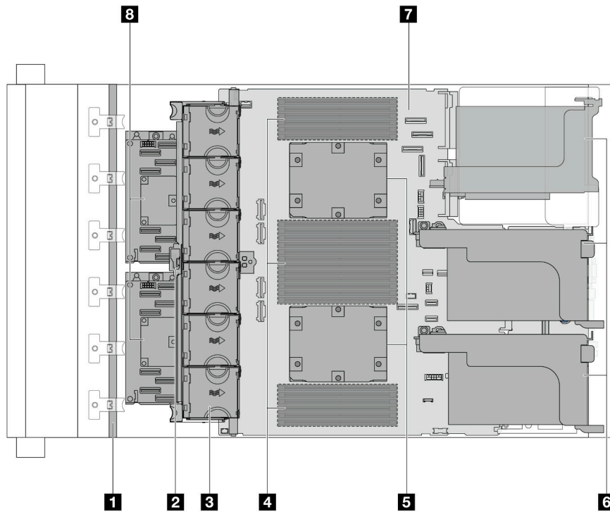
図9. 標準ヒートシンクのある上面図
