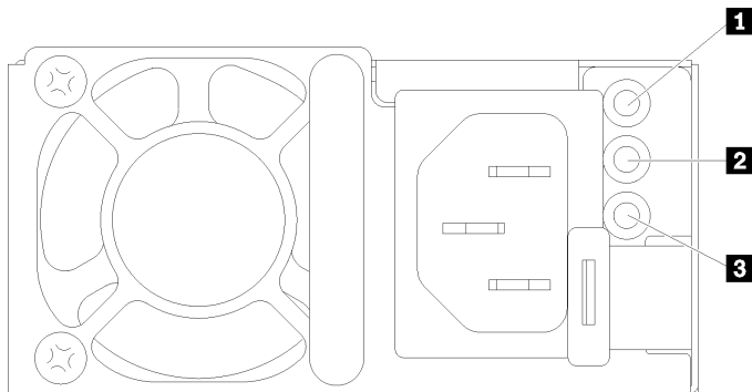
図 18. パワー・サプライ LED
