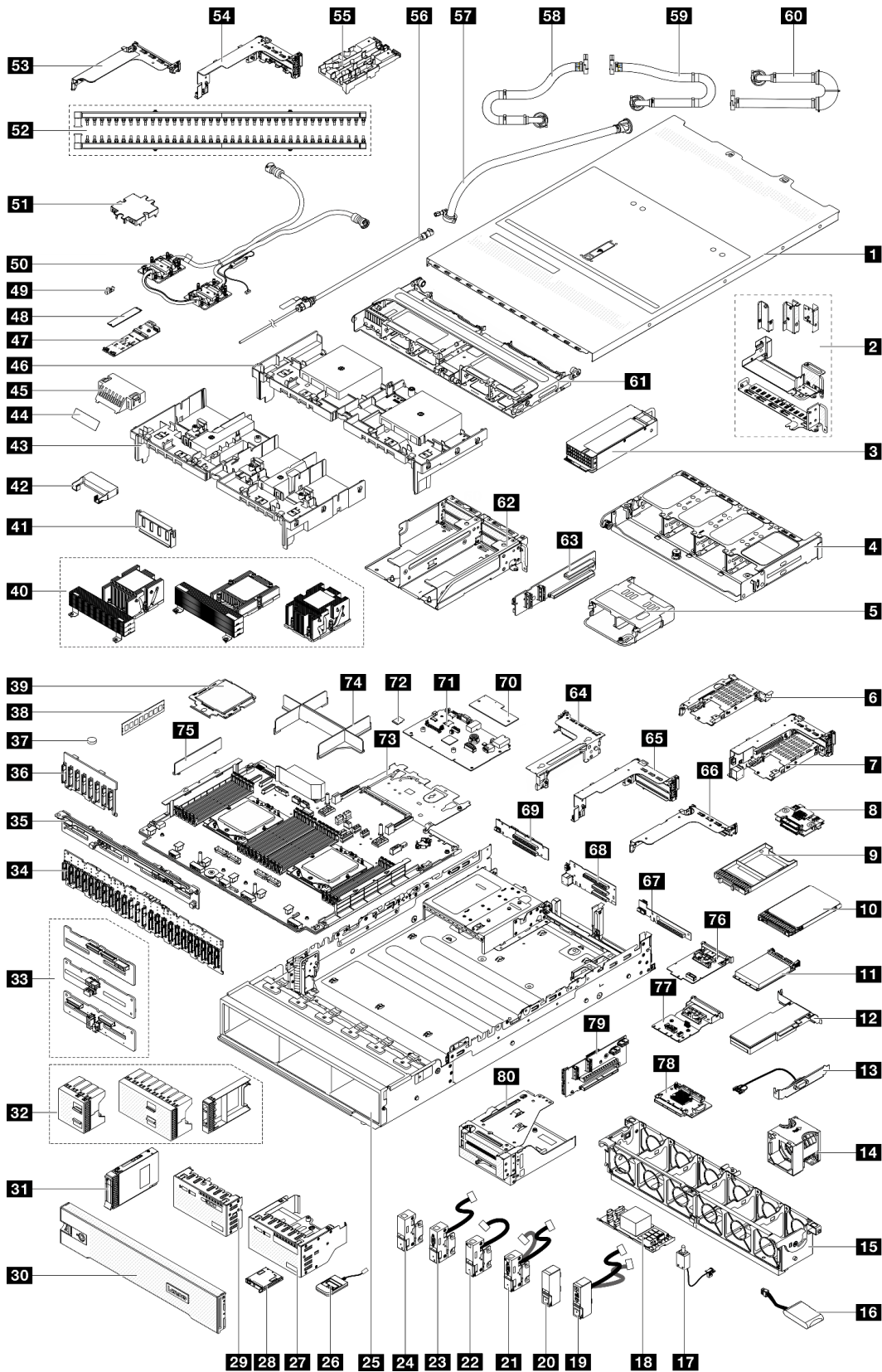
図 21. サーバー・コンポーネント (2.5 型ドライブ・ベイのシャーシ)
