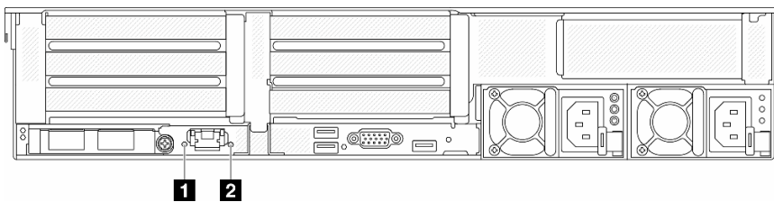
図 16. 背面システム LED
