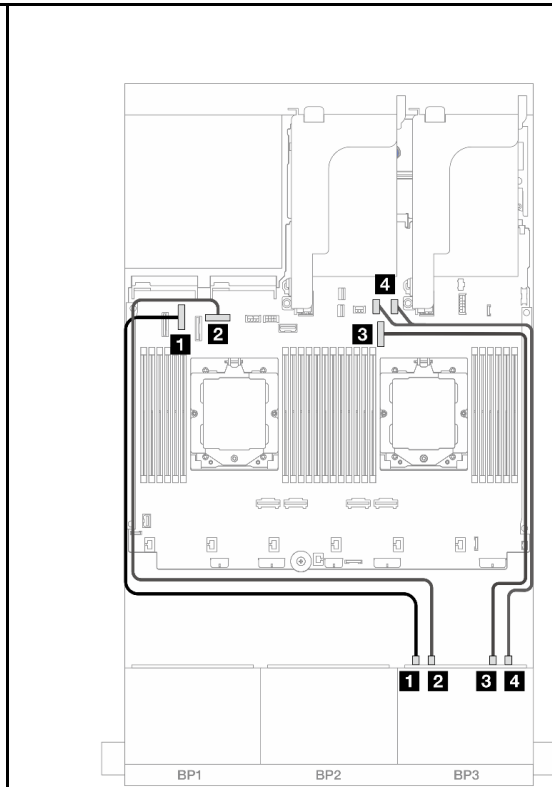
図 521. NVMe ケーブル配線
