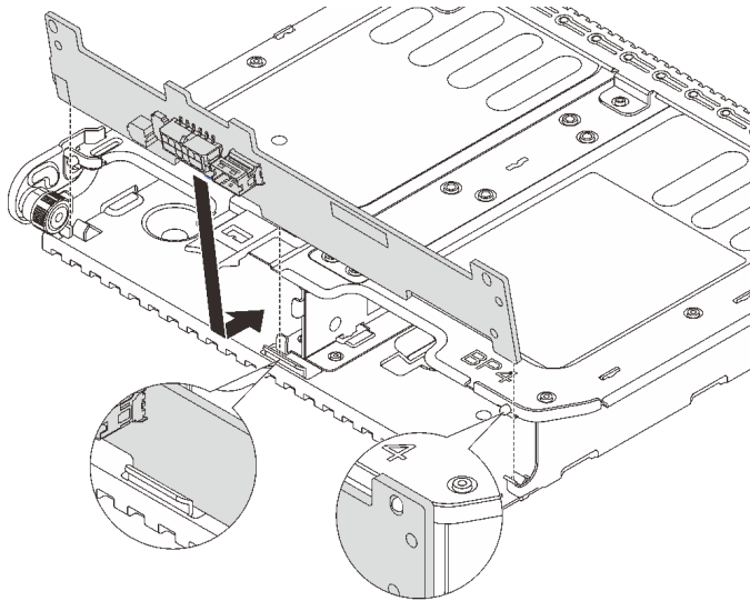
図 253. 2 x 3.5 型背面ドライブ・バックプレーンの取り付け
