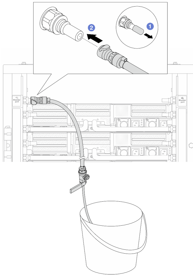
図 154. 供給側へのブリーダー・キットの取り付け
