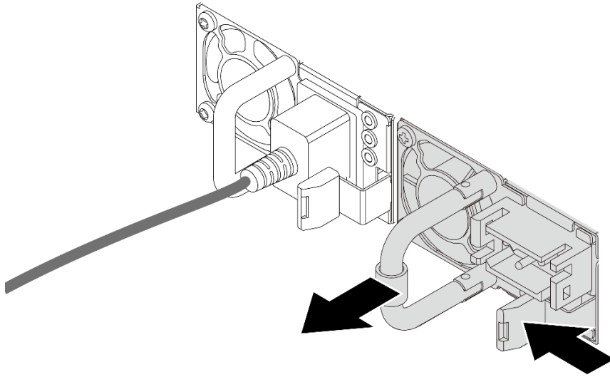
図 190. パワー・サプライ・ユニットの取り外し
