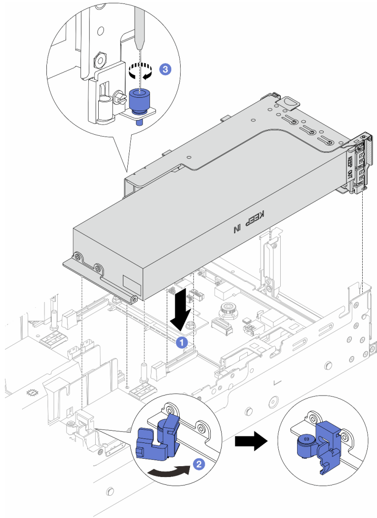
図 93. ライザー 1 アセンブリーへの GPU アダプターの取り付け
