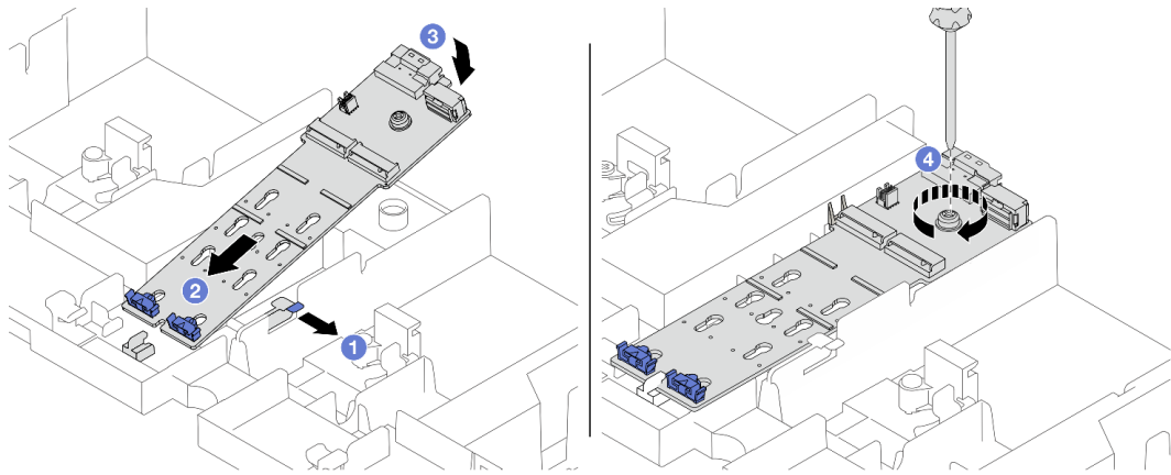
図 124. M.2 バックプレーンのエアール・バッフルへの取り付け
