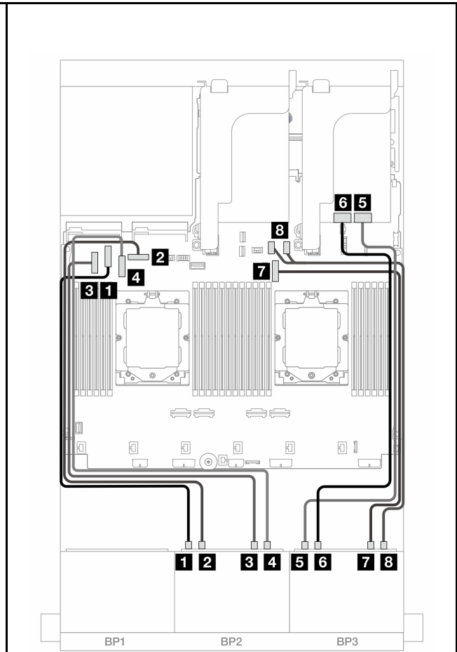
図 502. NVMe ケーブル配線
