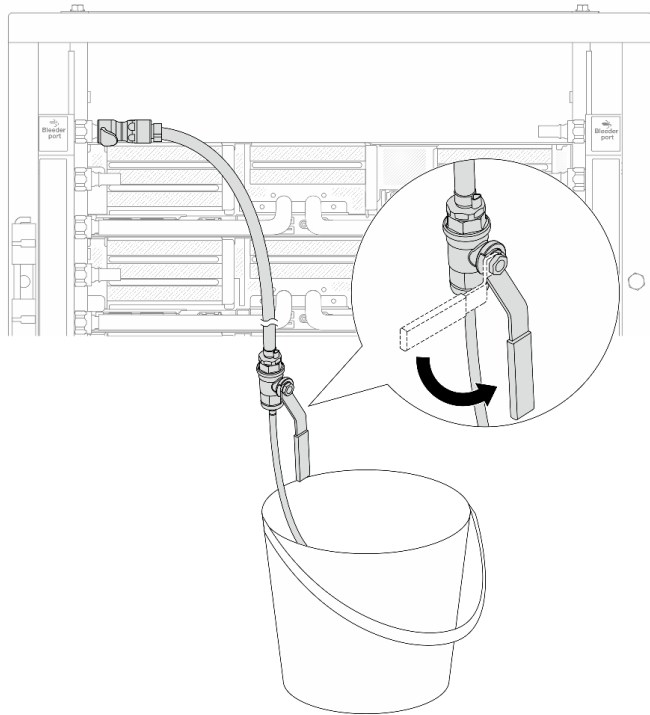
図 156. 供給側のブリーダのバルブを開く
