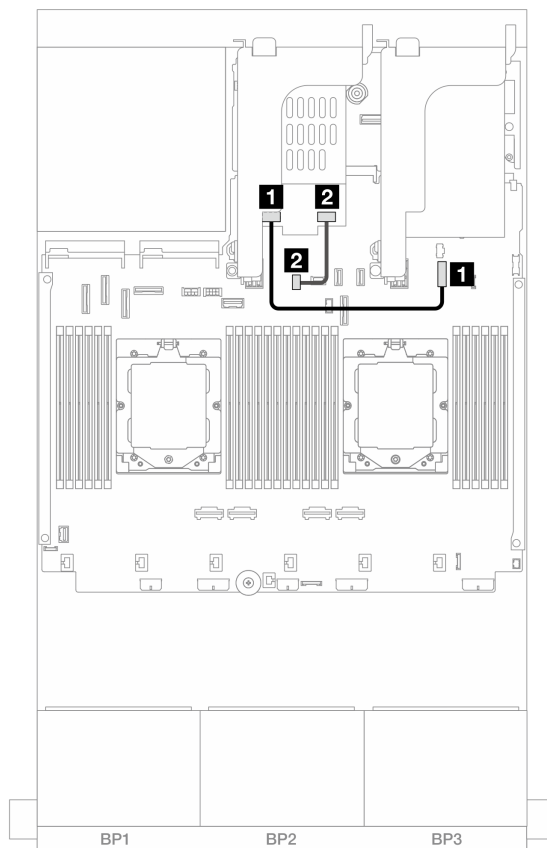
図 328. 7 mm RAID SATA/NVMe 2 ベイ・バックプレーン用ケーブルの配線
