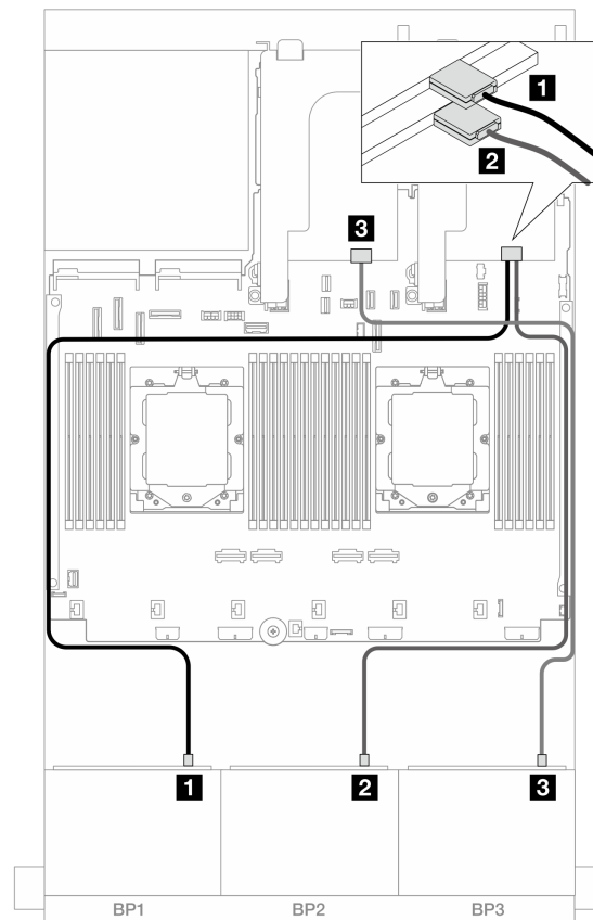
図 438. 8i アダプターへの SAS/SATA ケーブル配線
