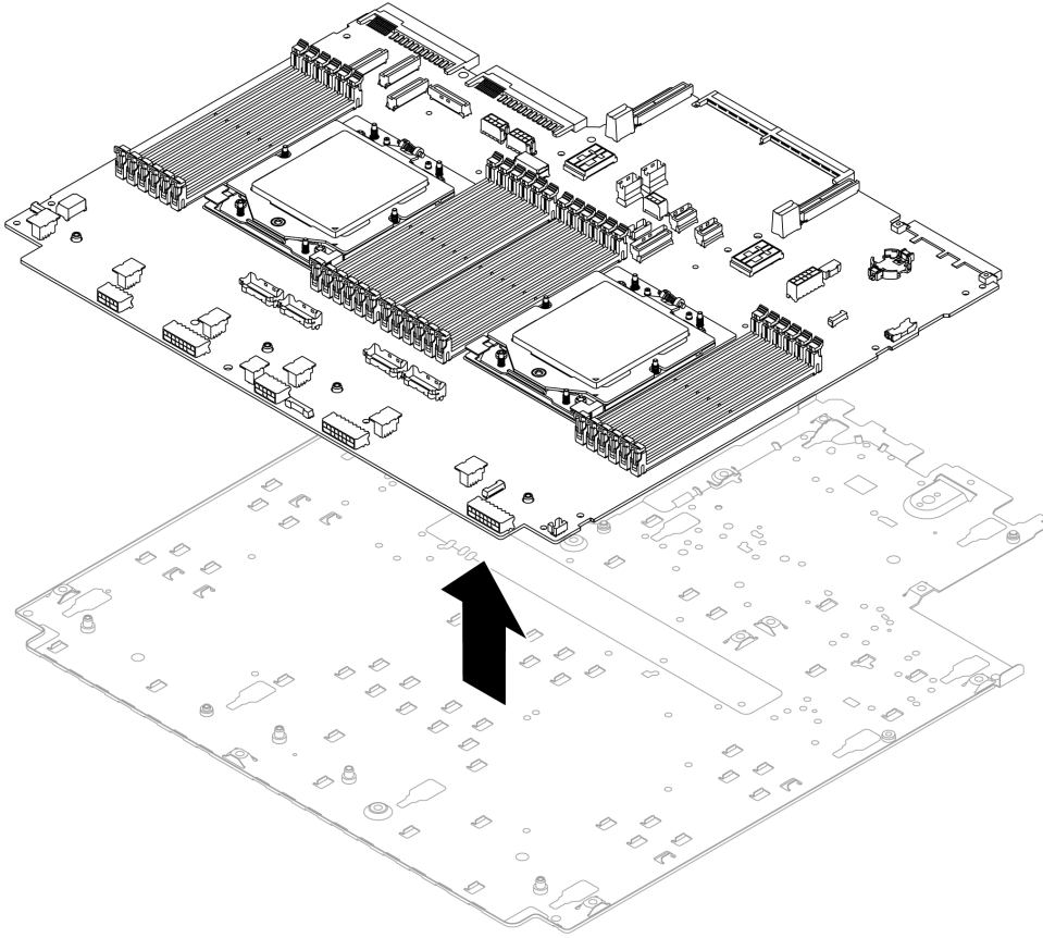
図 602. 保持用シート・メタルからのプロセッサ・ボードの分離
