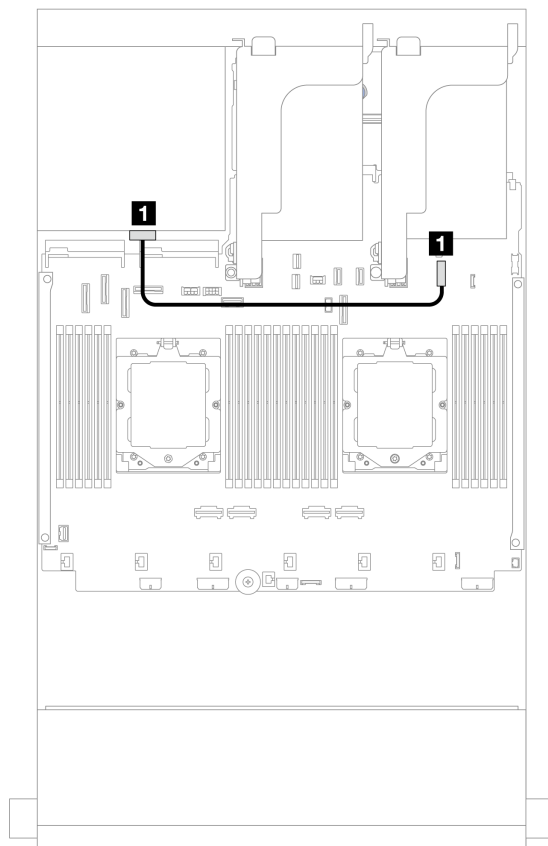
図 584. 背面バックプレーン電源ケーブルの配線
