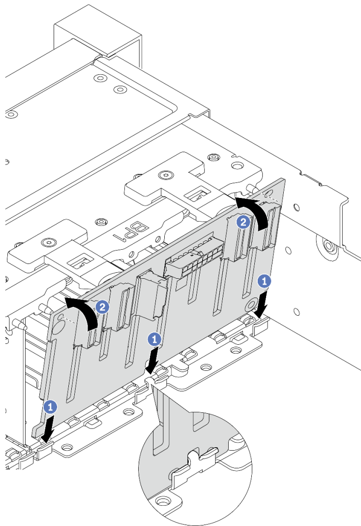
図 73. 8 ベイ・ドライブ・バックプレーンの取り付け
