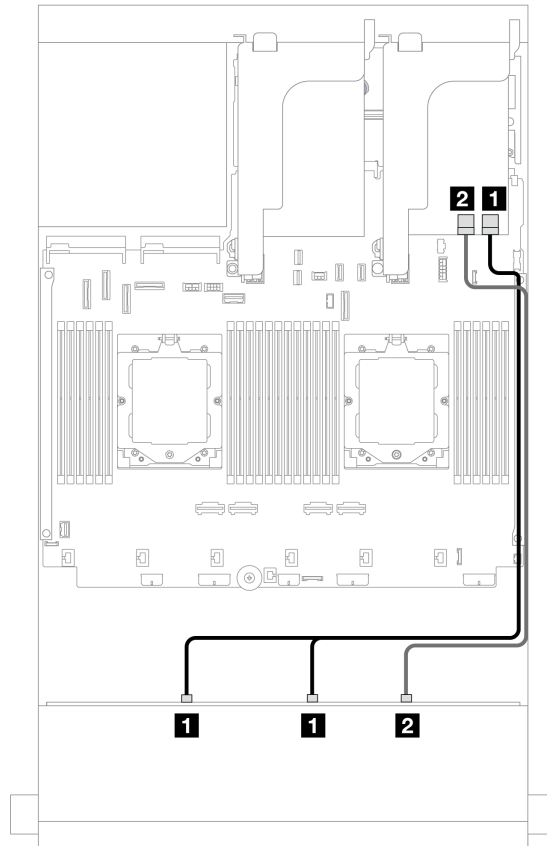
図 546. 1 つの 16i RAID/HBA アダプターへのケーブル配線
