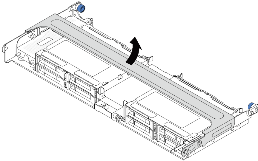
図 221. 中央ドライブ・ケージのハンドルを開く
