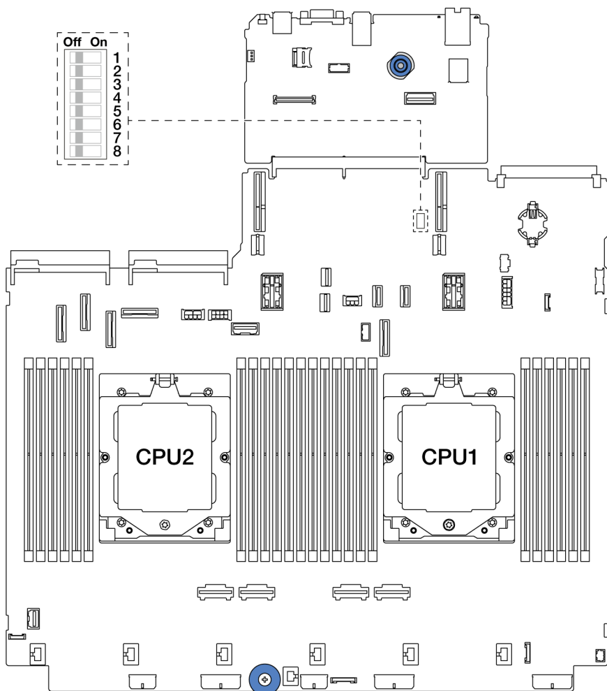
図13. システム・ボード・アセンブリー上のスイッチ・ブロック
