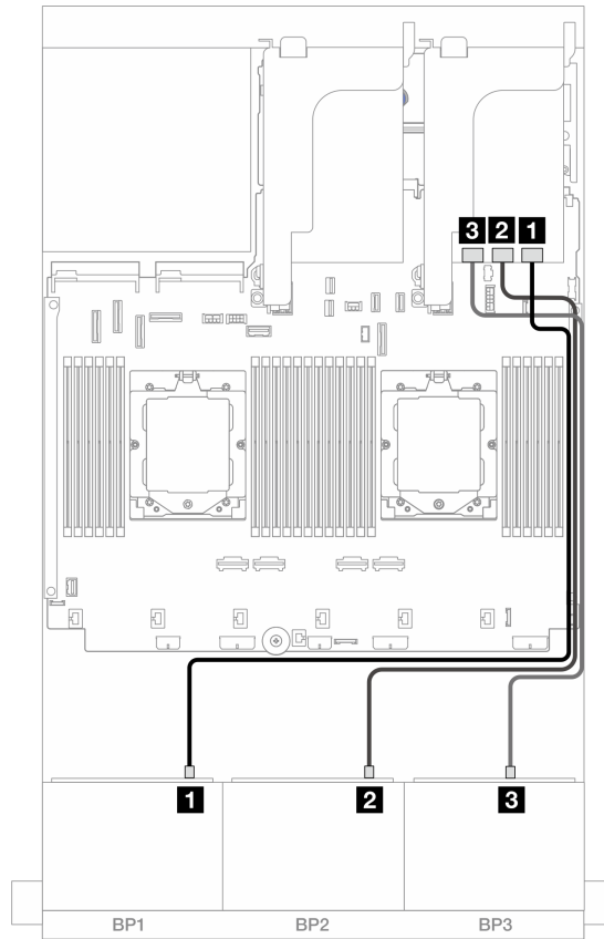
図 503. 32i アダプターへの SAS/SATA ケーブル配線
