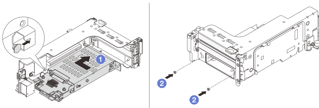
図 240. 7mm ドライブ・ケージのライザー・アセンブリーへの取り付け
