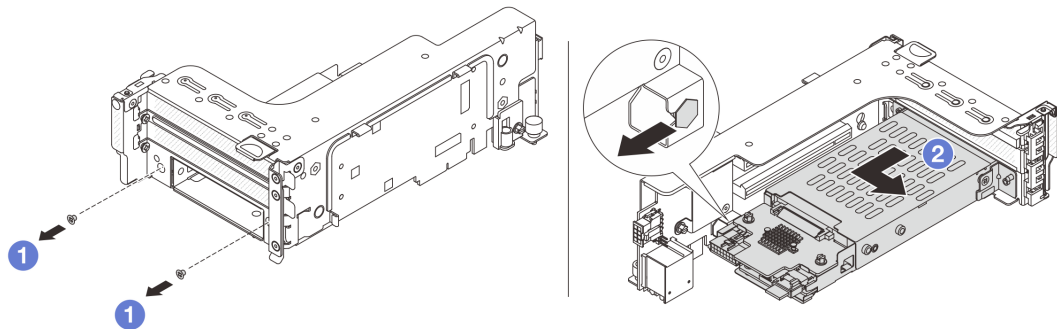
図 234. ライザー・アセンブリーからの 7mm ドライブ・ケージの取り外し
