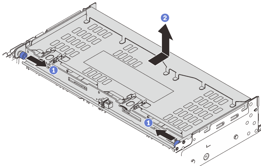
図 255. 4 x 3.5 型背面ドライブ・ケージの取り外し
