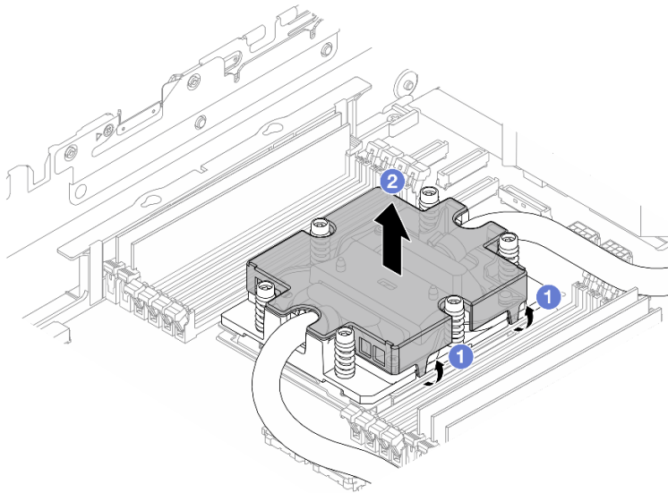
図 598. コールド・プレート・カバーの取り外し
