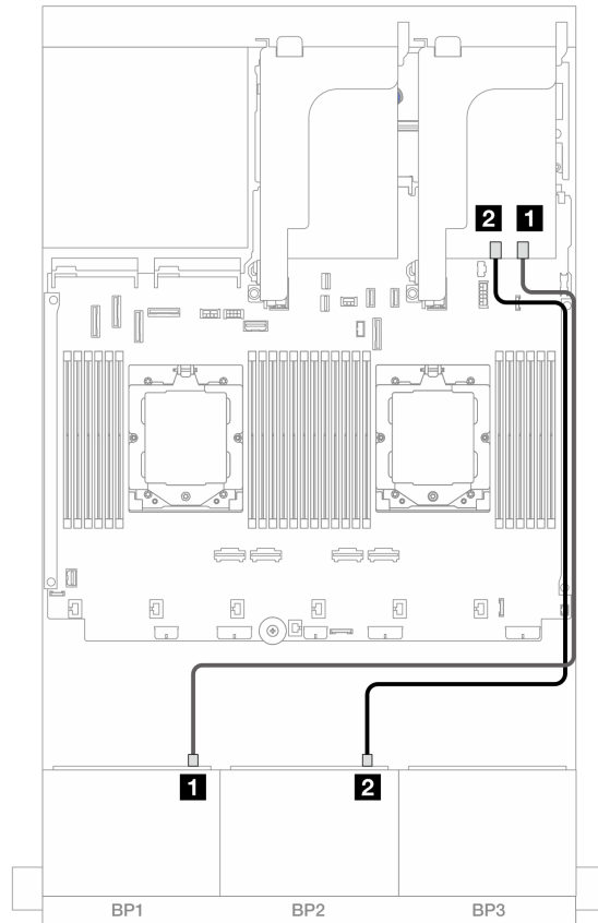
図 390. 16i RAID/HBA アダプターへの SAS/SATA ケーブル配線
