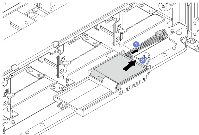
図 214. スーパーキャップ・ホルダーからの RAID フラッシュ電源モジュールの取り外し
