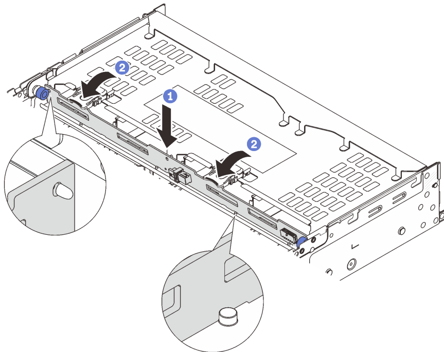
図257. 4 x 3.5 型背面ドライブ・バックプレーンの取り付け
