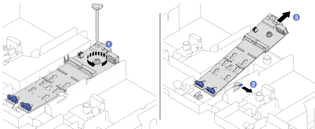
図 121. M.2 バックプレーンのエアー・バッフルからの取り外し
