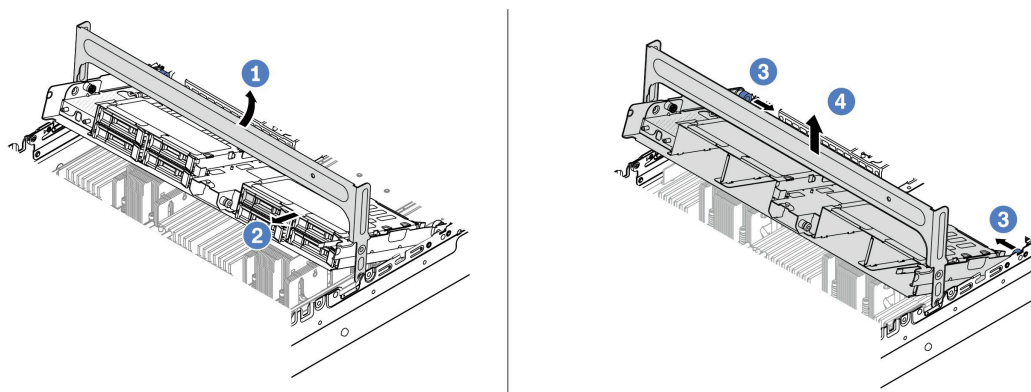
図 183. 中央ドライブ・ケージの取り外し
