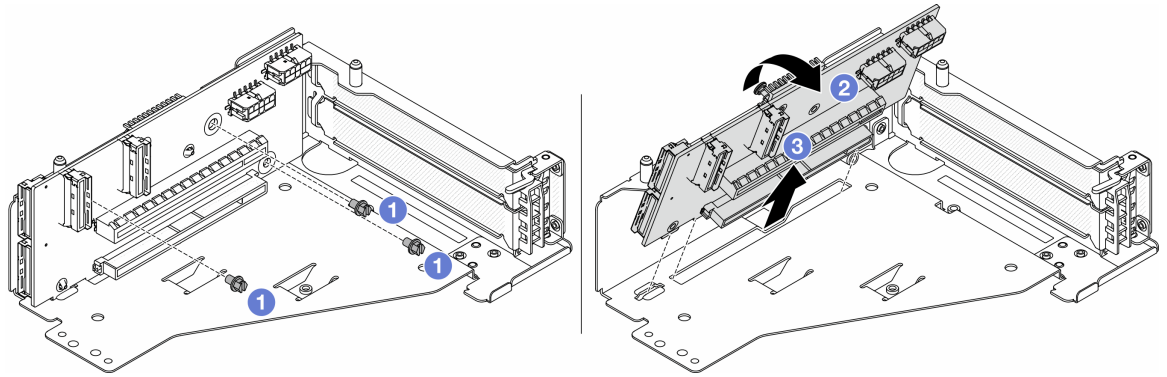
図 41. ライザー 5 ケージからのライザー・カードの取り外し
