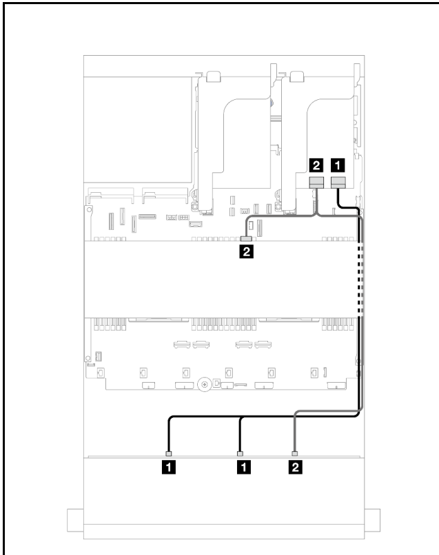
図 558. 前面/中央バックプレーン信号ケーブル配線
