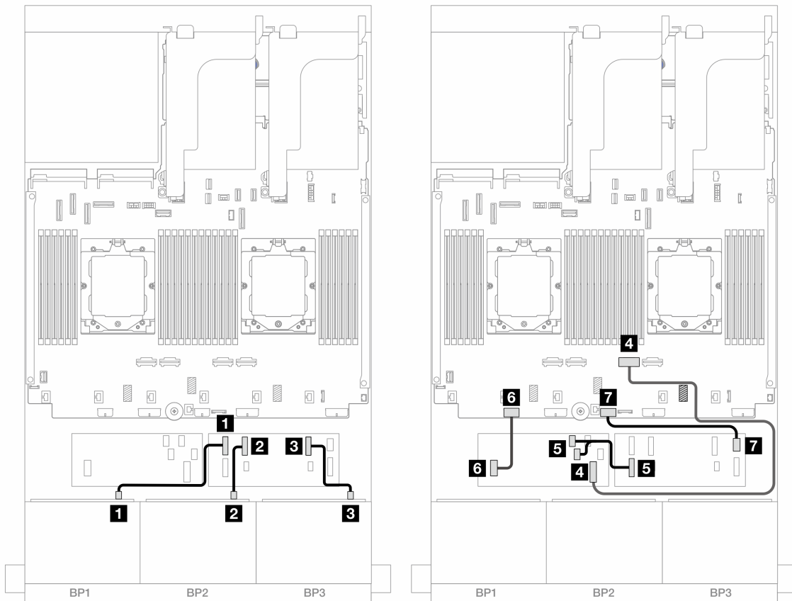
図 454. CFF エクスパンダーおよび CFF 16i アダプターへの SAS/SATA ケーブル配線
