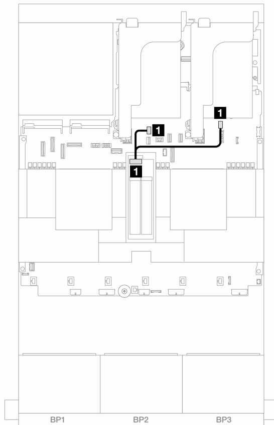
図 338. M.2 RAID SATA/NVME 2 ベイ・バックプレーンのケーブル配線
