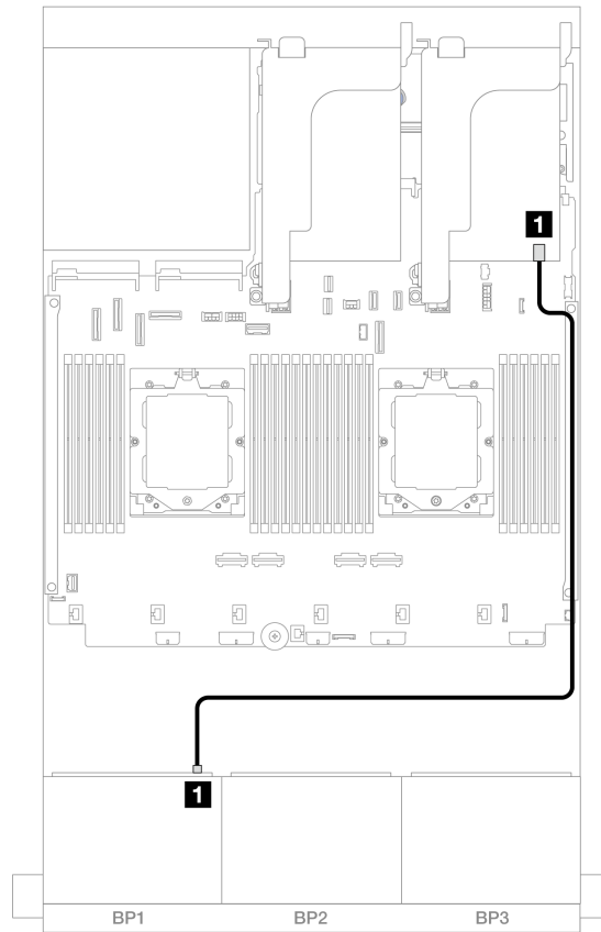
図 362. 8i/16i RAID/HBA アダプターへの SAS/SATA ケーブル配線
