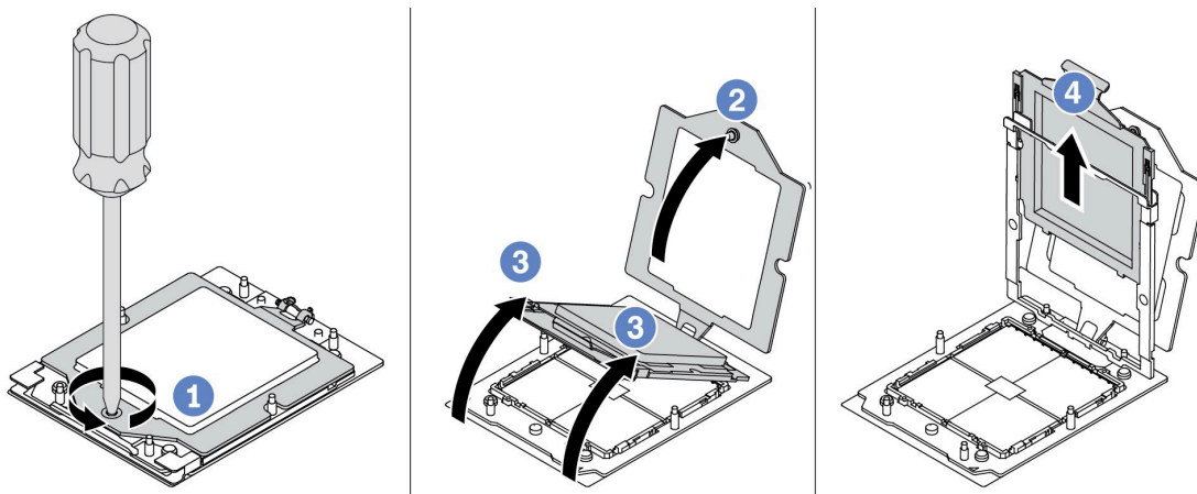
図 196. プロセッサの取り外し
