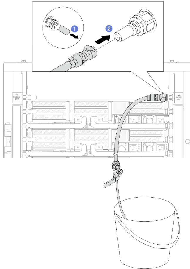
図 174. リターン側へのブリーダー・キットの取り付け
