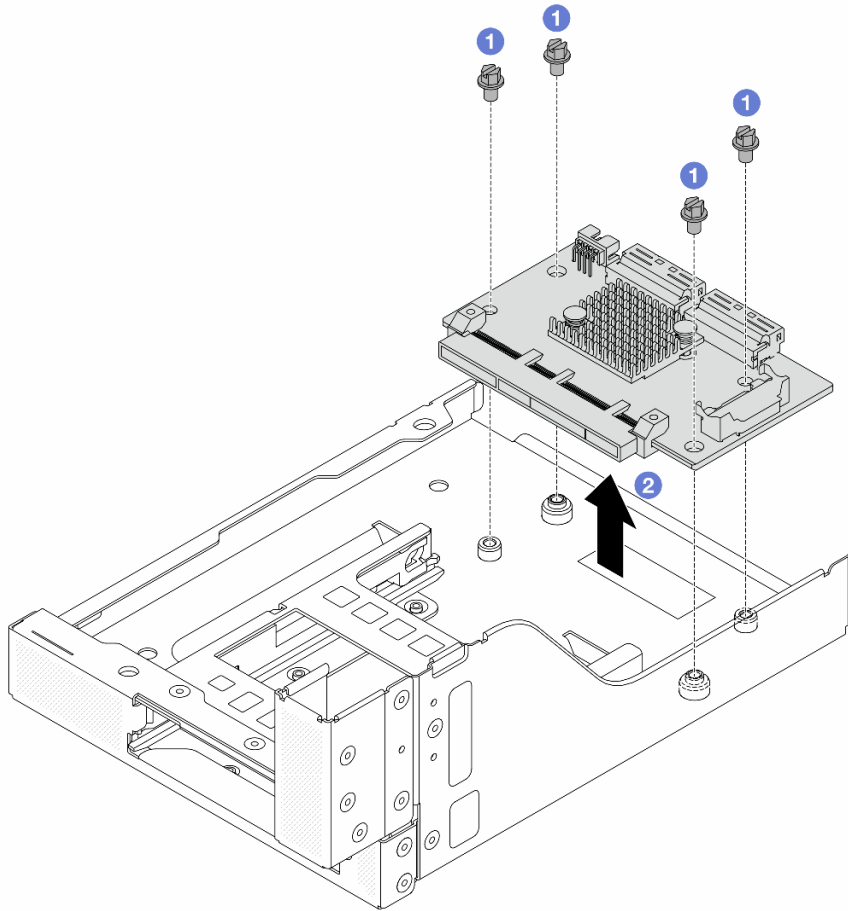
図 43. 前面 OCP 変換コネクタ・カードの取り外し
