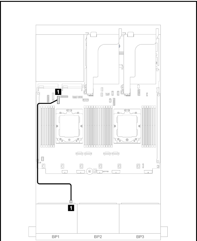
図 383. NVMe ケーブル配線
