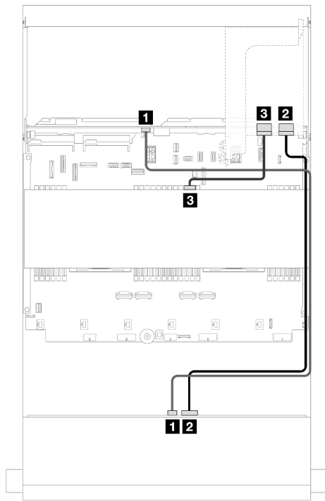
図 585. バックプレーン信号ケーブル配線
