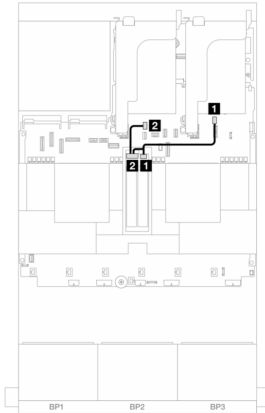
図 337. M.2 x1 RAID NVMe 2 ベイ・バックプレーンのケーブル配線
