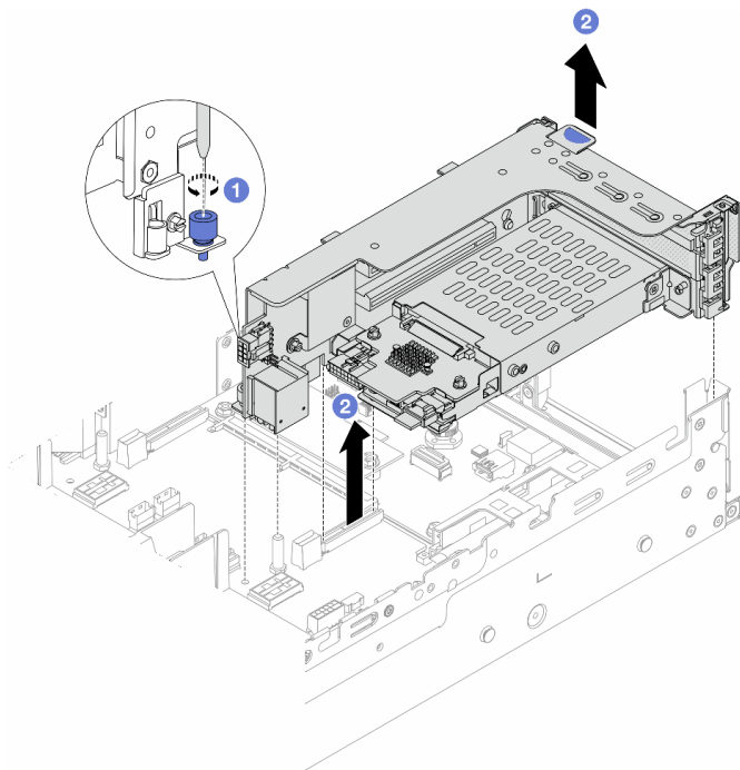
図 232. 2FH+7mm SSD ライザー・ケージの取り外し
