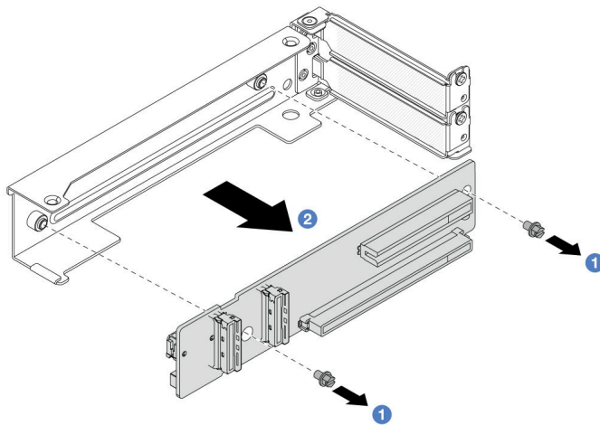
図 273. 4LP ライザー 3/4 ケージからのライザー・カードの取り外し
