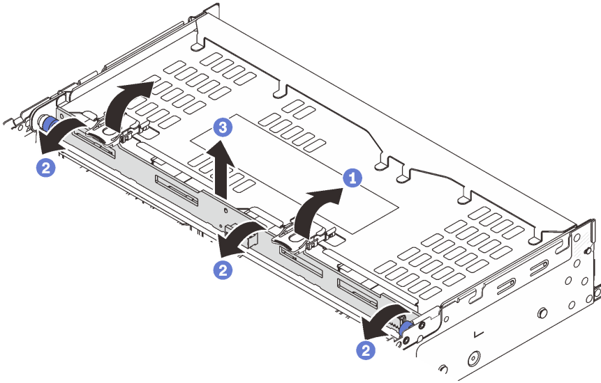
図 256. 4 x 3.5 型背面ドライブ・バックプレーンの取り外し
