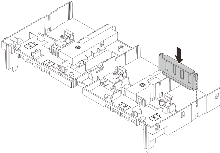
図94. GPU エア・バッフル・フィルターの取り付け
