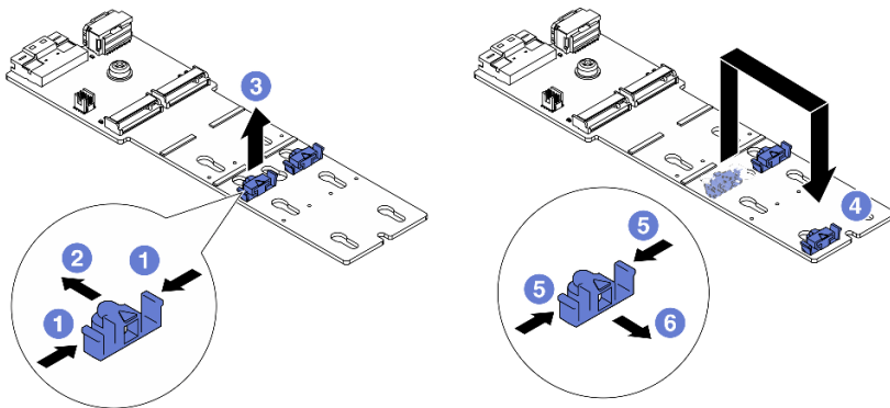
図 115. M.2 保持器具の調整
