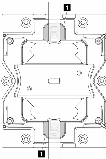
図 597. 漏れやすいエリア
