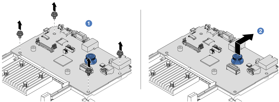
図 599. システム I/O ボードのプロセッサ・ボードからの取り外し
