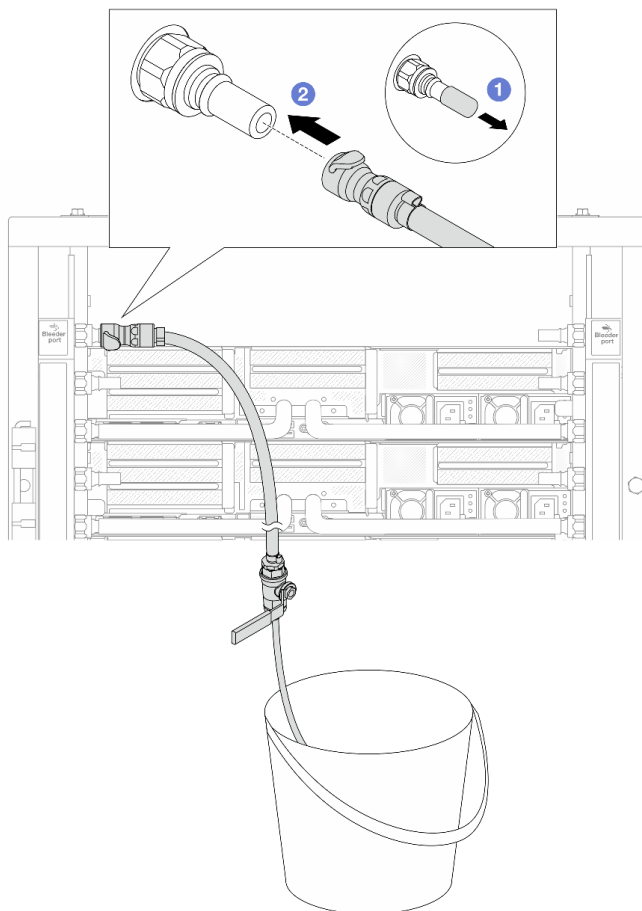
図 171. 供給側へのブリーダー・キットの取り付け
