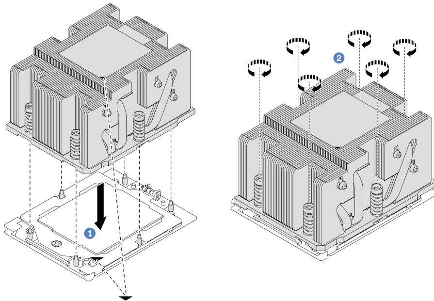
図 201. 標準ヒートシンクの取り付け
