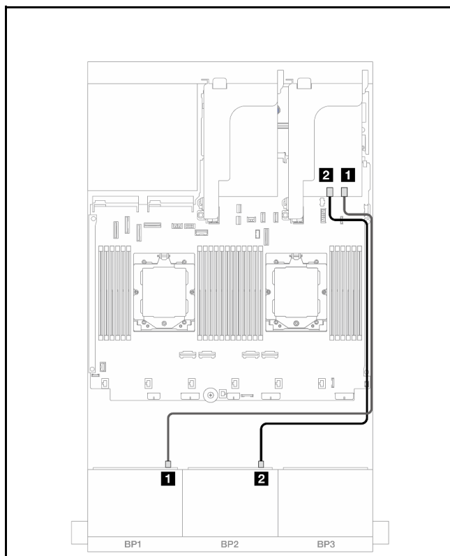
図 395. 前面バックプレーンのケーブル配線
