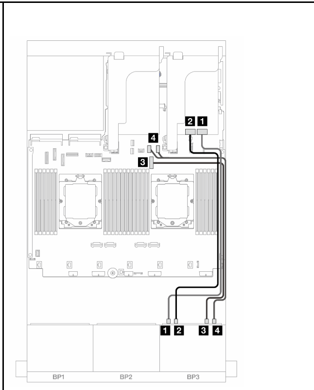
図 531. NVMe ケーブル配線
