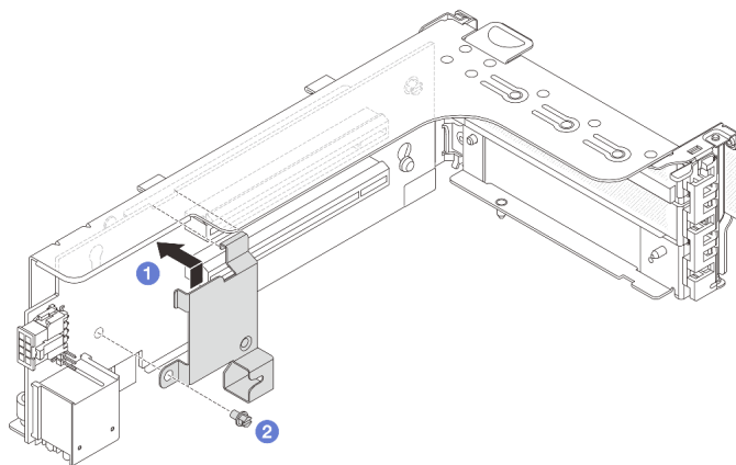
図 239. 7mm ドライブ・ケージの固定クリップの取り付け
