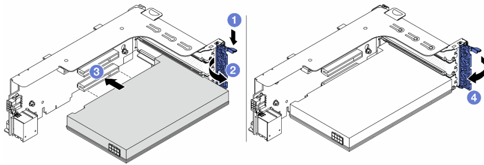
図 277. PCIe アダプターのライザー 1 または 2 アセンブリーへの取り付け
