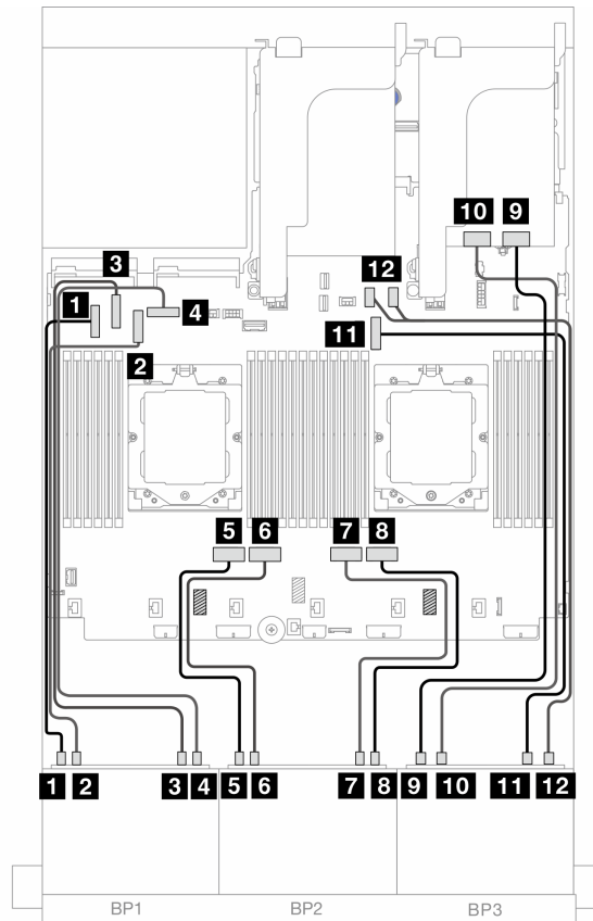
図 496. オンボード・コネクタおよびリタイマー・カードへの NVMe ケーブル配線
