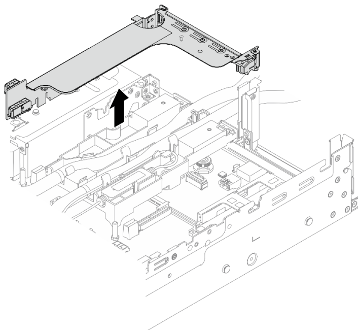
図 101. 1FH ライザー・ケージの取り外し
