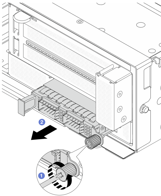
図 50. 前面 OCP モジュールの取り外し
