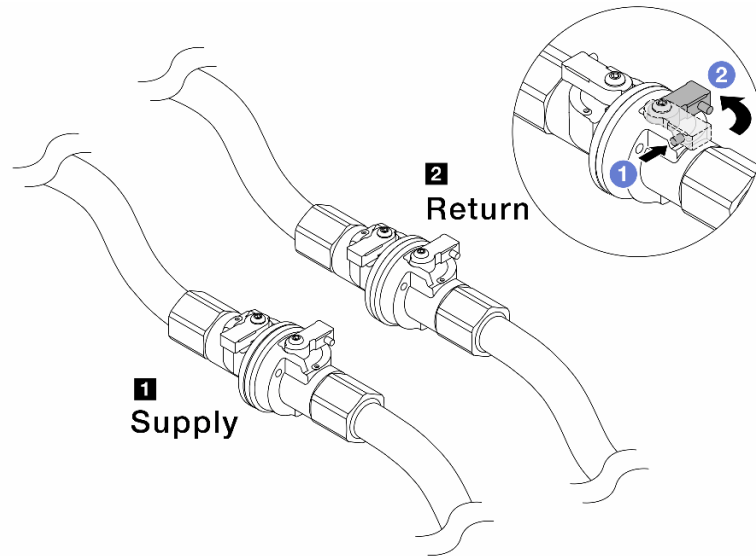
図160. ボール・バルブを閉じる
