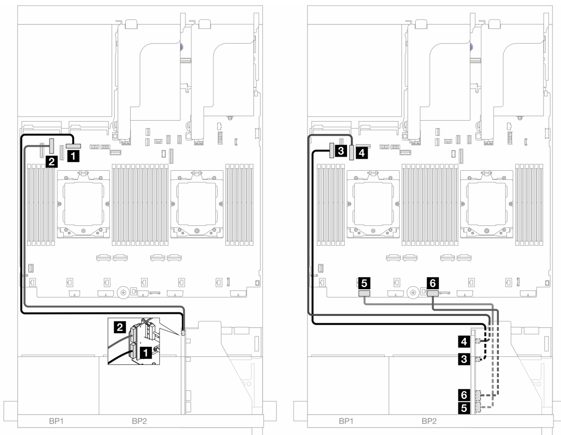
図 355. ライザー 3/4 のない構成のケーブル配線
