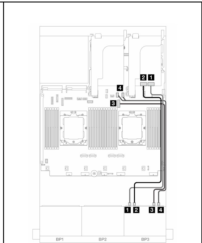
図511. NVMe ケーブル配線
