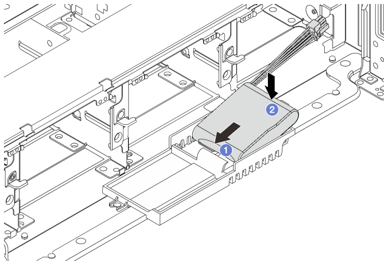
図 217. スーパーキャップ・ホルダーへの RAID フラッシュ電源モジュールの取り付け
