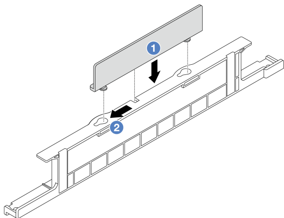
図 35. 2U ケーブル壁ブラケットの取り付け
