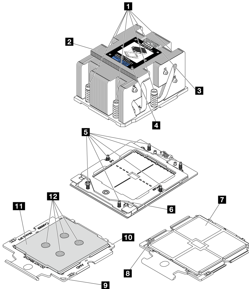
図 193. プロセッサおよびヒートシンク・コンポーネント
