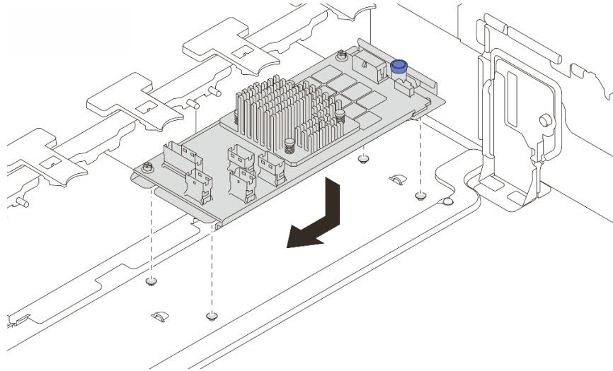
図97. 内蔵 CFF アダプターの取り付け
