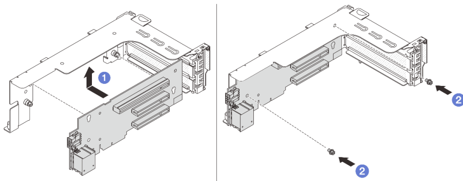
図274. ライザー 1 または 2 ケージへのライザー・カードの取り付け
