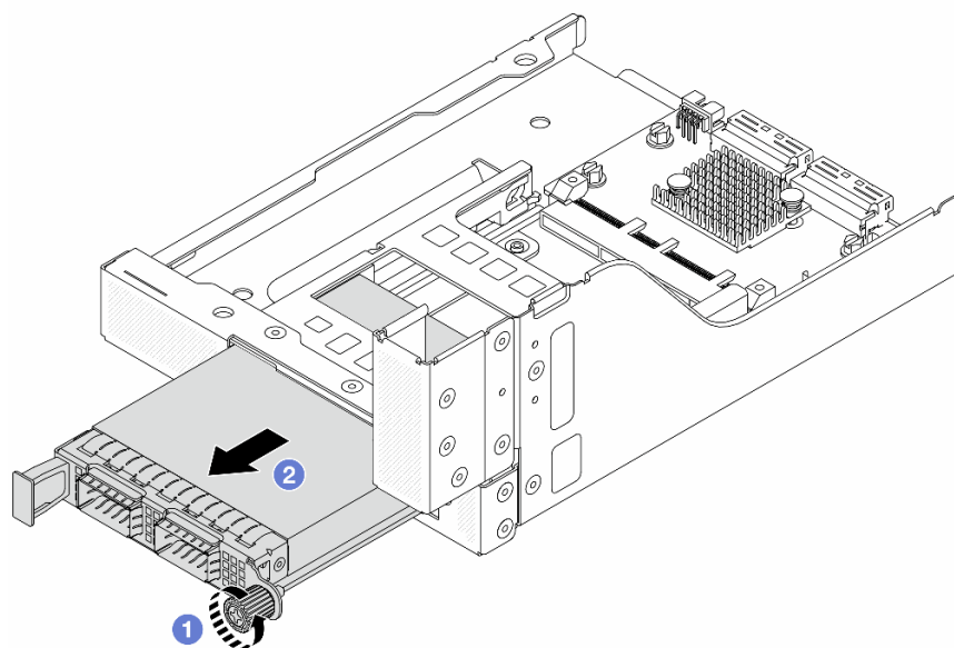
図 54. OCP モジュールの取り外し
