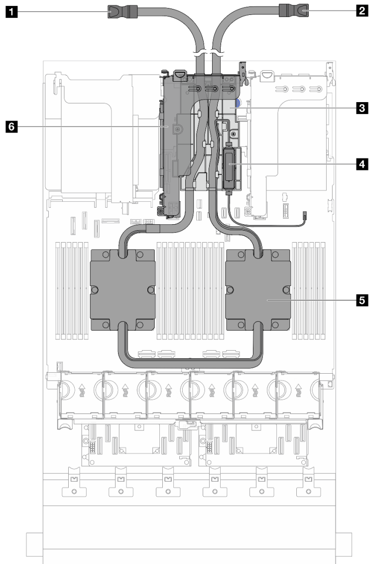
図 10. DWCM を使用した上部図
