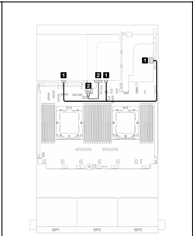
図 458. 背面バックプレーンのケーブル配線
