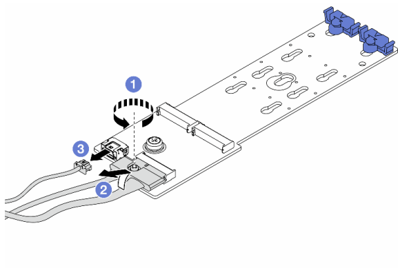
図 119. M.2 x1 RAID NVMe 2 ベイ・バックプレーンからのケーブルの取り外し
