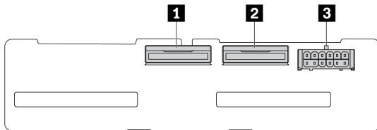
図 319. 4 x 2.5 型 NVMe バックプレーン・コネクタ
