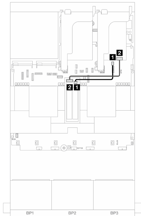
図 336. RAID ケーブル配線
