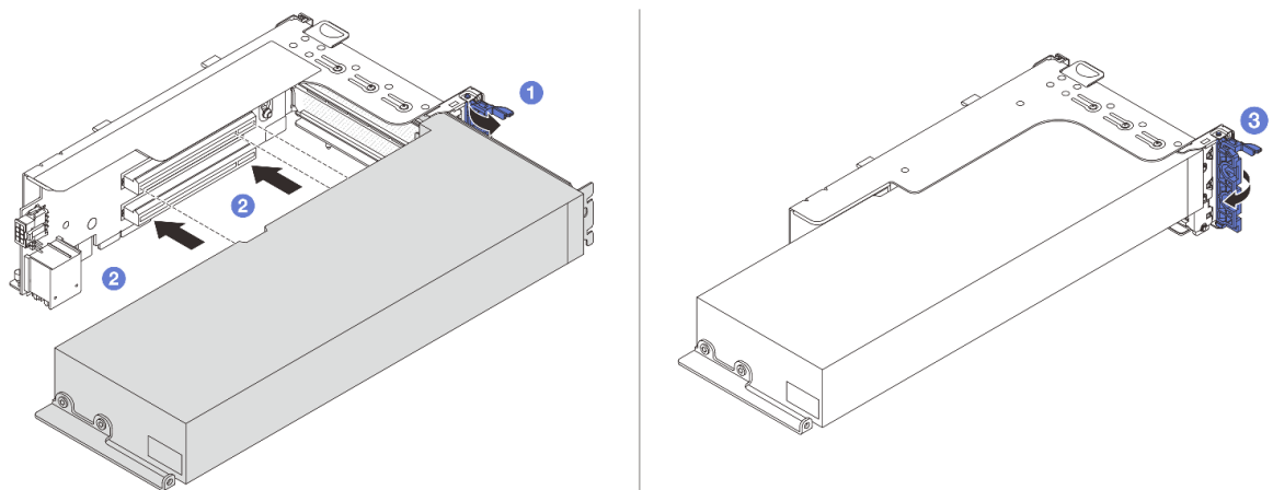
図 91. GPU アダプターの取り付け
