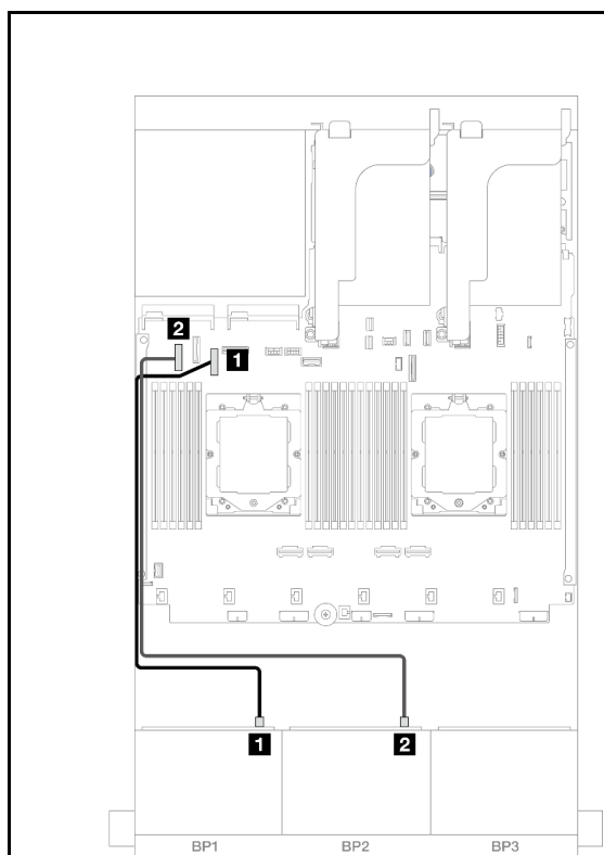
図 388. 2つのプロセッサが取り付けられた場合のケーブル配線
