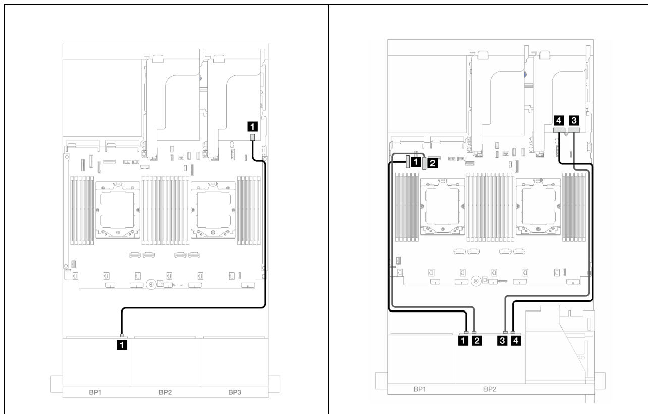
図 431. SAS/SATA ケーブル配線
