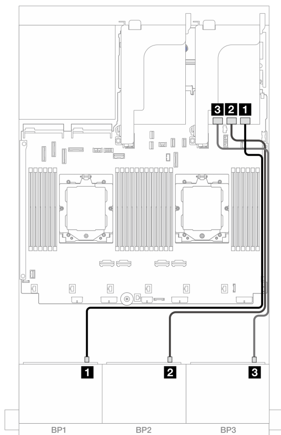
図 477. 32i アダプターへの SAS/SATA ケーブル配線
