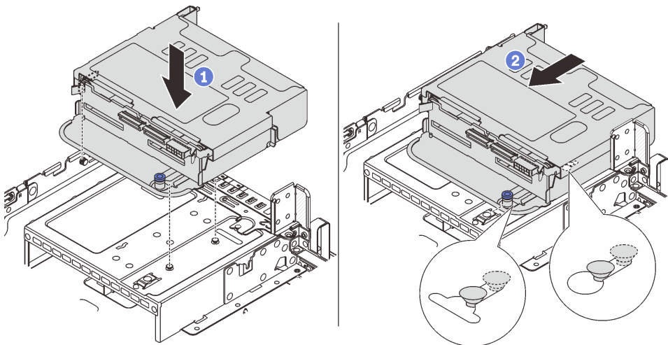
図 246. 4 x 2.5 型背面ドライブ・ケージの取り付け
