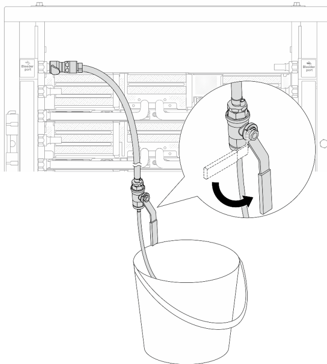
図 177. 供給側のブリーダーのバルブを開く
