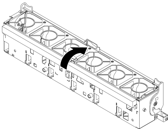
図 98. ファン・ケージの回転
