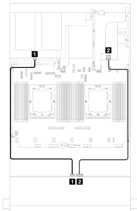
図 580. 前面/背面バックプレーン信号ケーブルの配線
