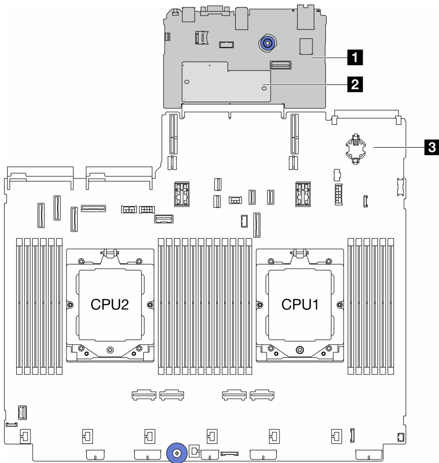
図 289. システム・ボード・アセンブリーのレイアウト
