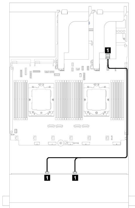
図 575. SAS/SATA ケーブル配線
