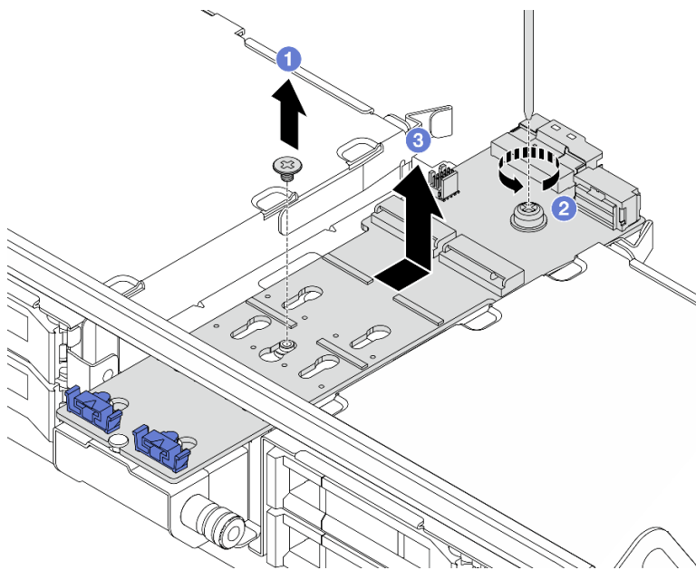
図 123. 中央ドライブ・ケージからの M.2 バックプレーンの取り外し
