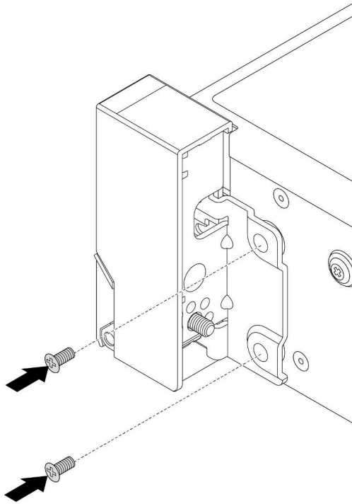
図 208. ねじの取り付け
