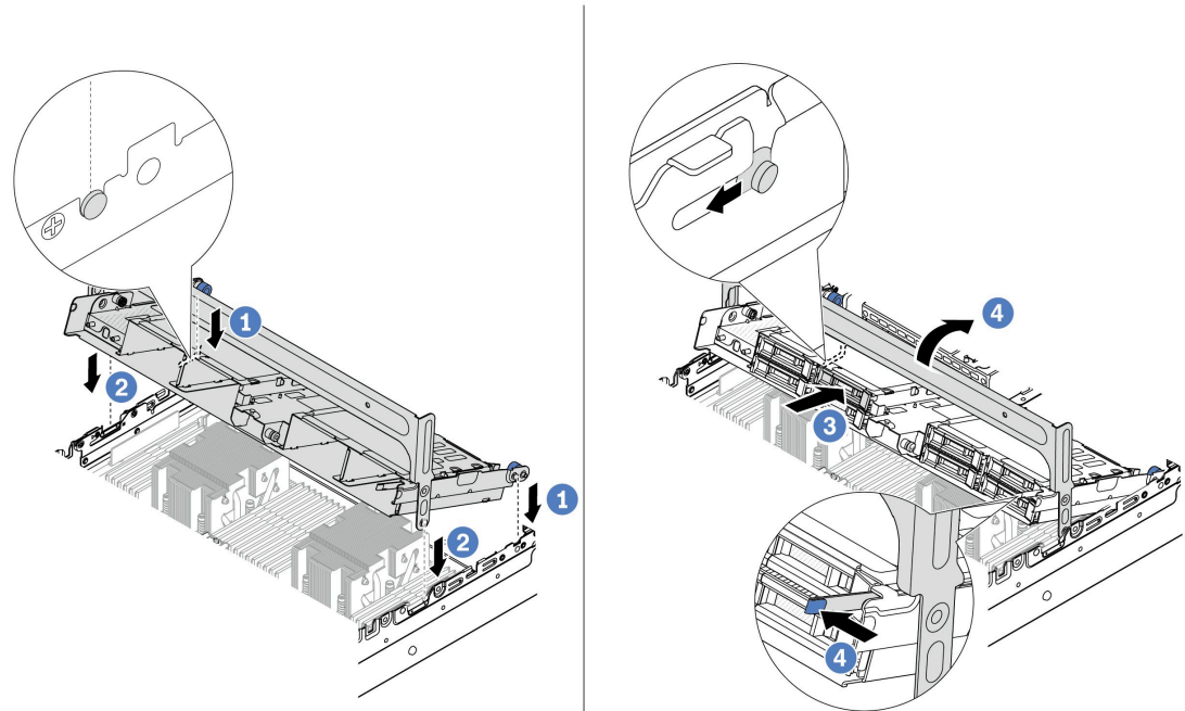
図 188. 中央ドライブ・ケージとドライブの取り付け
