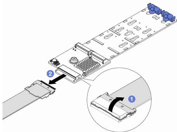
図 120. M.2 RAID SATA/NVME 2 ベイ・バックプレーンからのケーブルの取り外し
