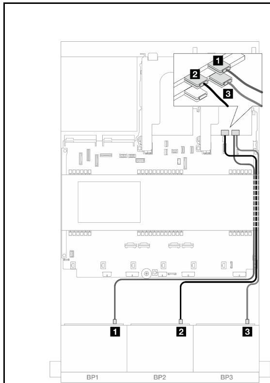
図 475. 前面バックプレーンのケーブル配線
