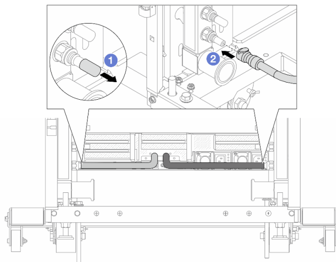
図 153. クイック・コネクト・プラグの取り付け
