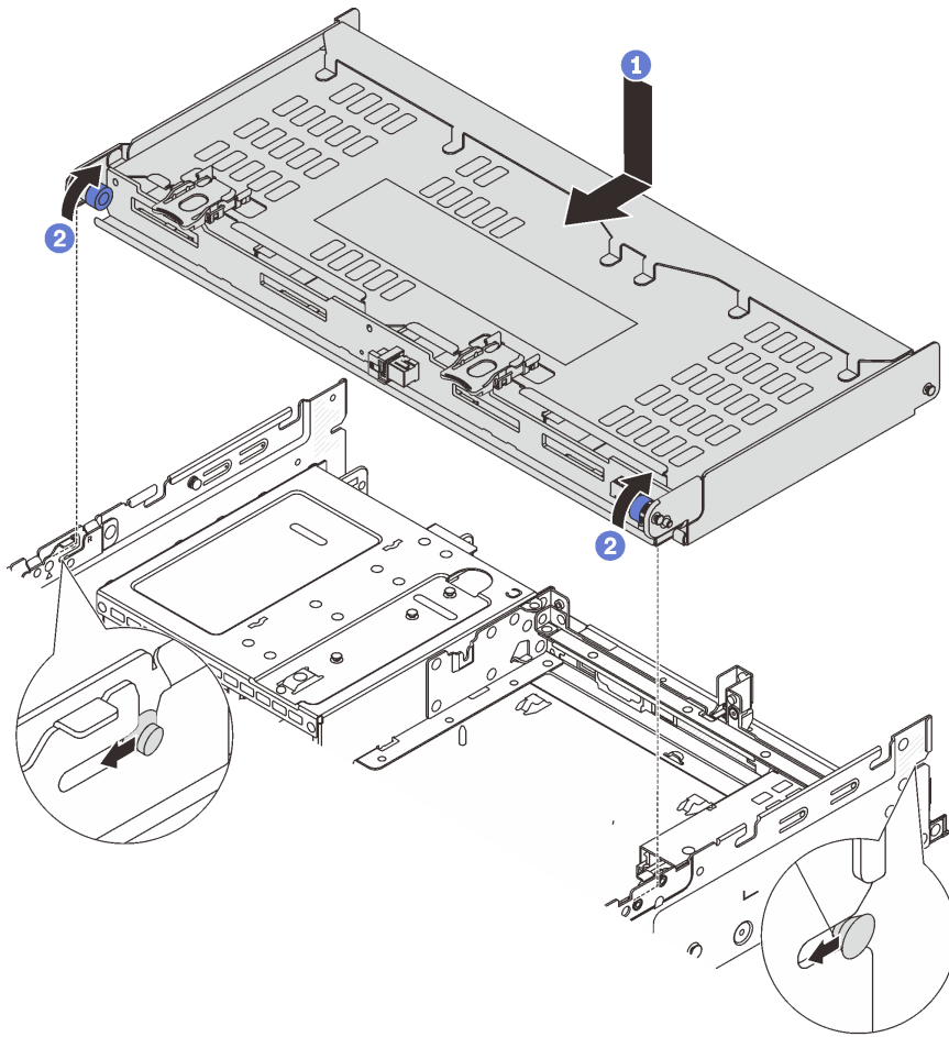
図 258. 4 x 3.5 型背面ドライブ・ケージの取り付け
