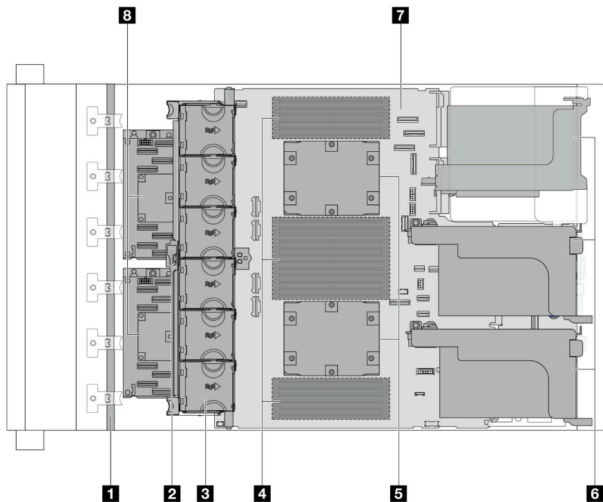
図9. 標準ヒートシンクのある上面図
