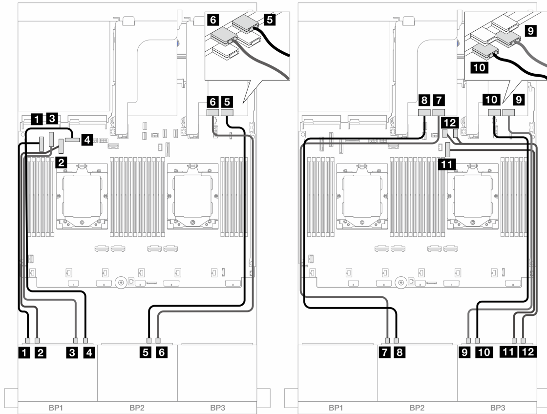
図 498. オンボード・コネクタおよびリタイマー・カードへの NVMe ケーブル配線
