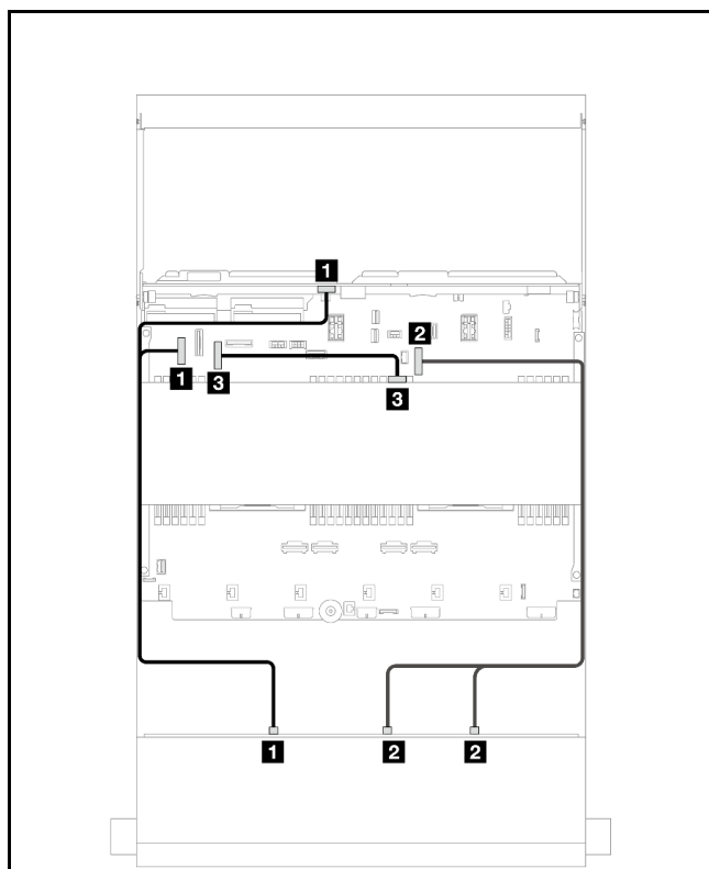
図 563. 前面/中央/背面バックプレーン信号ケーブル配線
