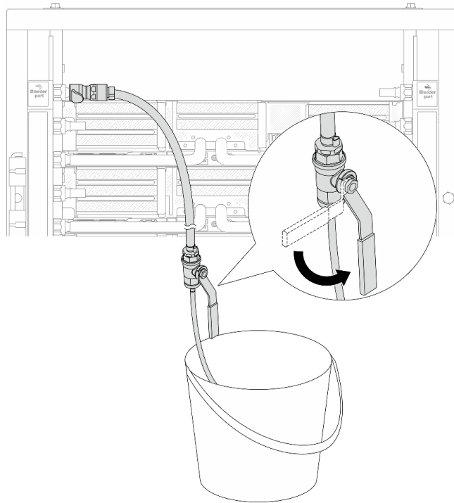
図 159. 供給側のブリーダーのバルブを開く
