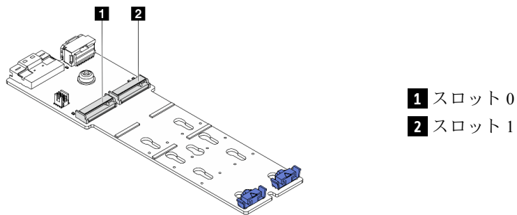
図 116. M.2 ドライブ・スロット
