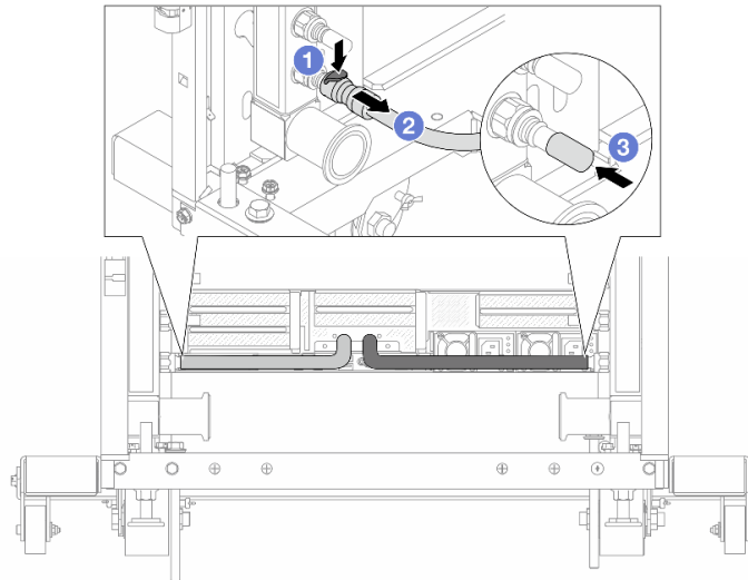
図 139. クイック・コネクット・プラグの取り外し
