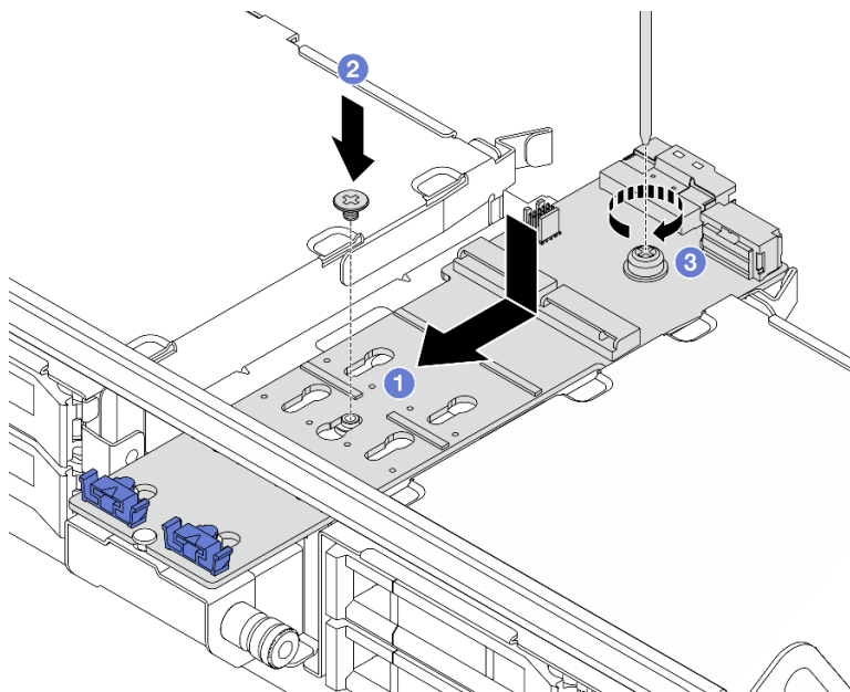
図 125. 中央ドライブ・ケージへの M.2 バックプレーンの取り付け
