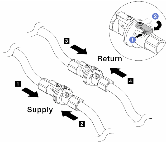
図 178. ボール・バルブを開く
