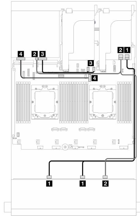
図 556. 1つのプロセッサが取り付けられた場合のケーブル配線
