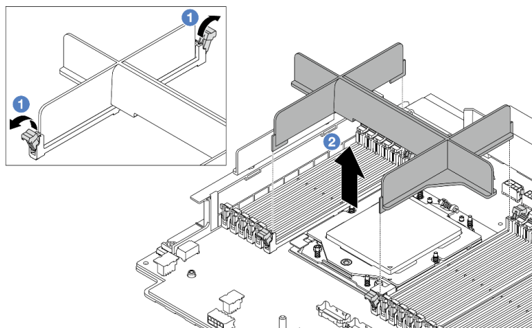
図 198. プロセッサ・フィラーの取り外し
