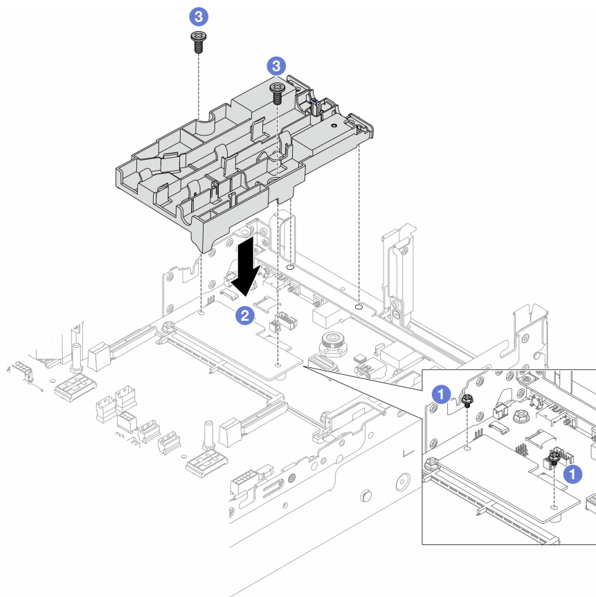
図 106. ホース・ホルダーの取り付け
