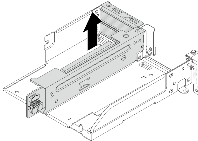
図 266. ライザー 3/4 アセンブリの取り外し
