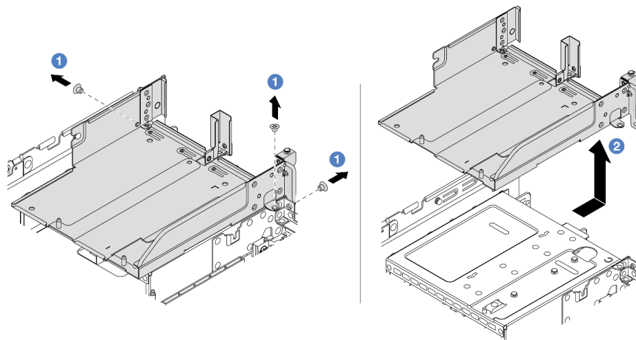
図 267. ライザー・ケージ・トレイの取り外し
