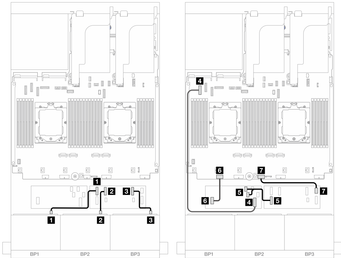
図 486. CFF エクスパンダーおよび CFF 16i アダプターへの SAS/SATA ケーブル配線
