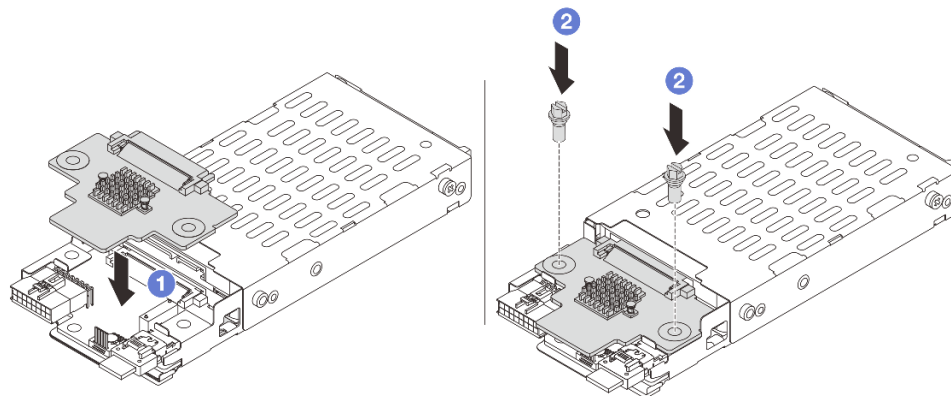
図 238. 7 mm ドライブ・バックプレートの取り付け (上部)
