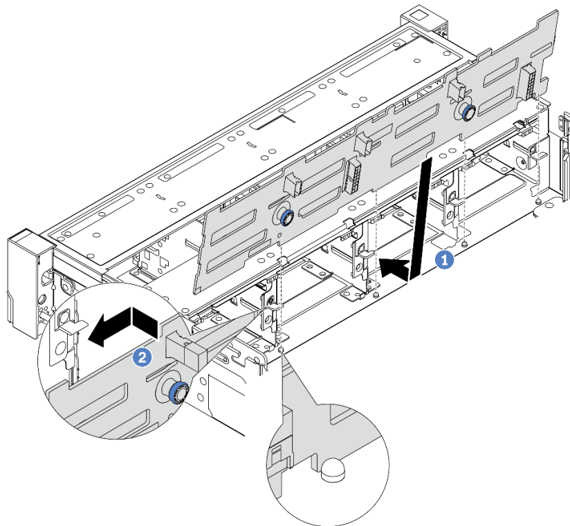
図 76. 3.5 型ドライブ・バックプレーンの取り付け
