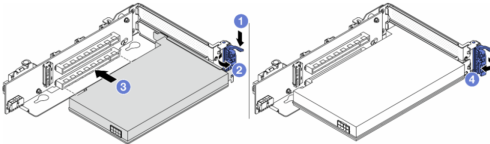
図 278. PCIe アダプターのライザー 3 アセンブリーへの取り付け
