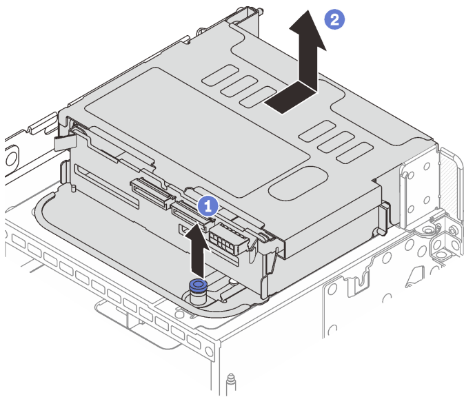
図 243. 4 x 2.5 型背面ドライブ・ケージの取り外し
