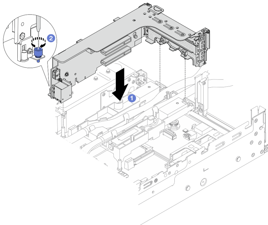
図 113. 3FH ライザー・ケージの取り付け
