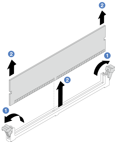
図 179. メモリー・モジュールの取り外し
