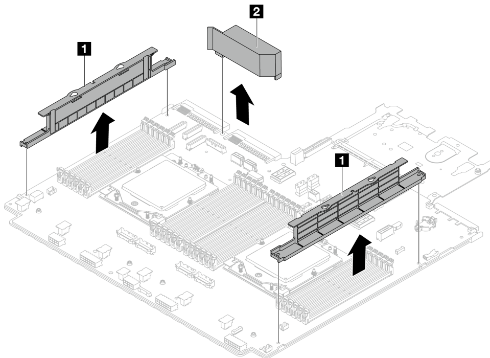
図601. プロセッサ・ボードからのコンポーネントの取り外し
