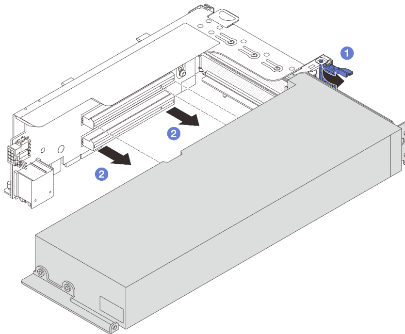
図 90. GPU アダプターの取り外し
