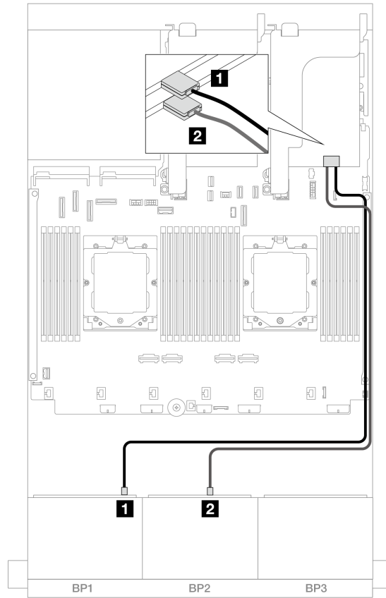
図 406. 8i アダプターへの SAS/SATA ケーブル配線
