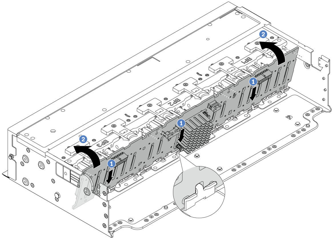
図 74. 24 ベイ・エキスパンダー・バックプレーンの取り付け
