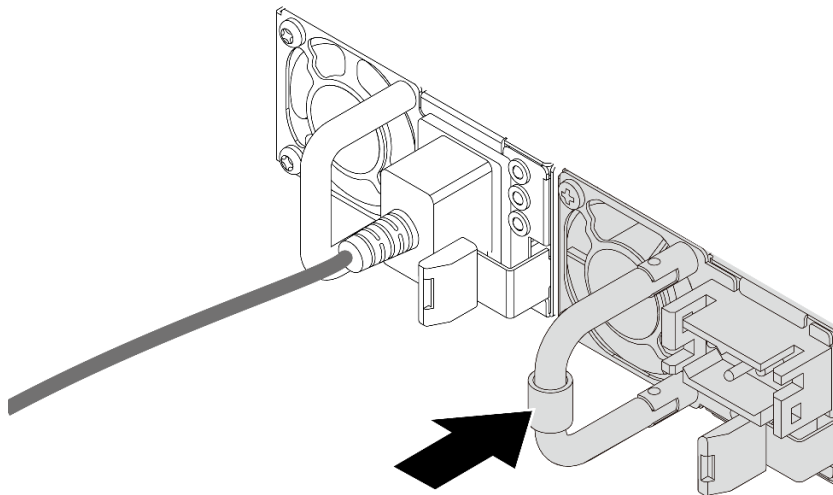
図 192. パワー・サプライ・ユニットを取り付けた後に:
