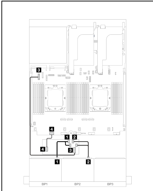
図 530. CFF アダプターのケーブル配線
