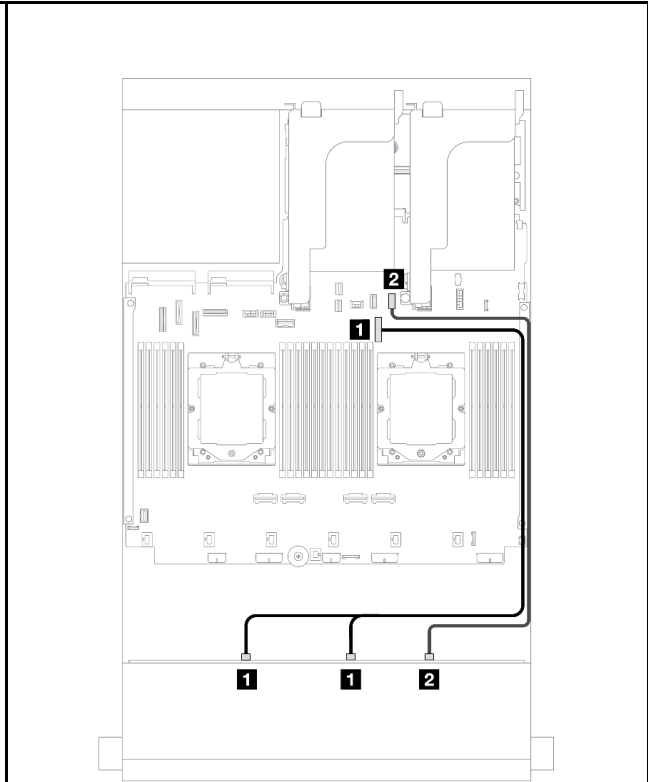
図 545. 1つのプロセッサが取り付け済みである場合のオンボード SATA コネクタへのケーブル配線
