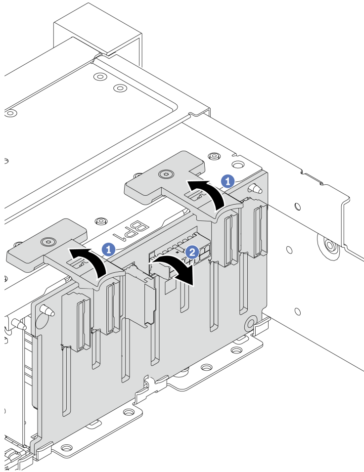
図70. 8ベイ・ドライブ・バックプレーンの取り外し
