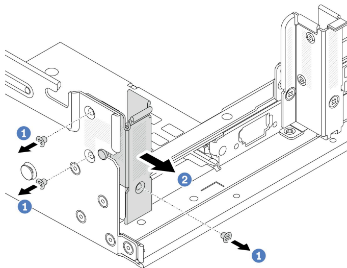
図 226. A1 背面壁ブラケットの取り外し (左)
