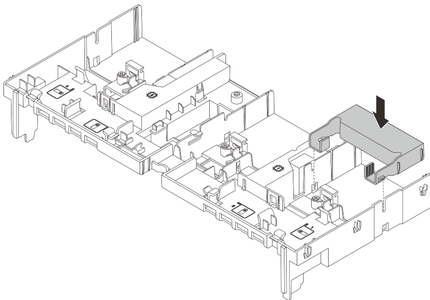
図92. アドオン・エアー・バッフル1の取り付け
