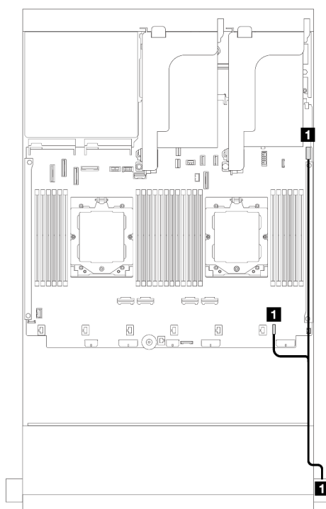
図 331. 前面オペレーター・パネルおよび USB コネクタ (右のラック・ラッチ)
