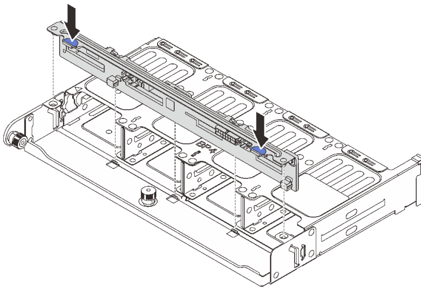
図 249. 8 x 2.5 型背面ドライブ・バックプレーンの取り付け
