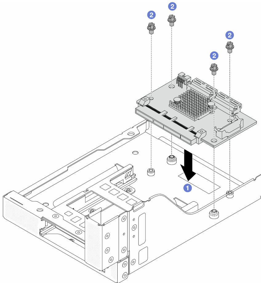
図 44. 前面 OCP 変換コネクタ・カードの取り付け
