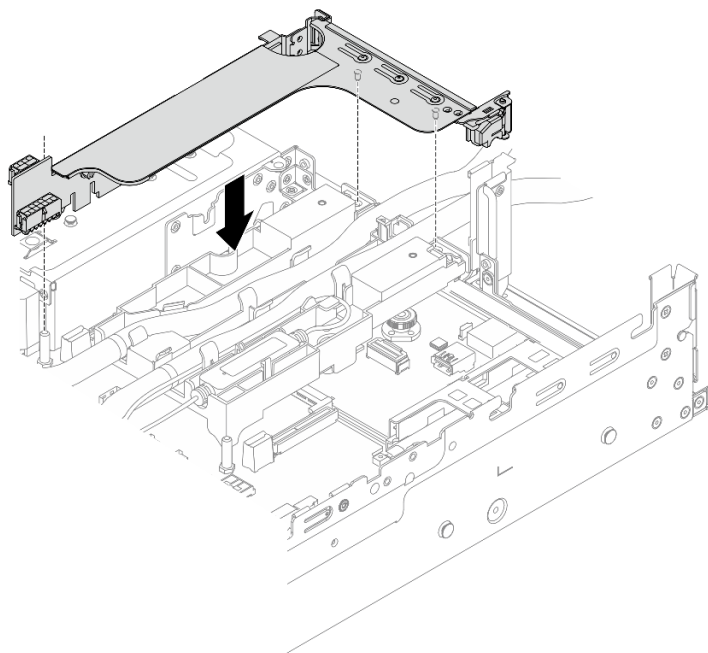
図 112. 1FH ライザー・ケージの取り付け
