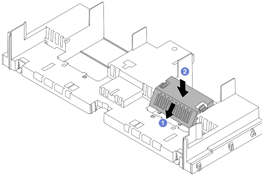
図32. エアー・バッフル・フィルターの取り付け
