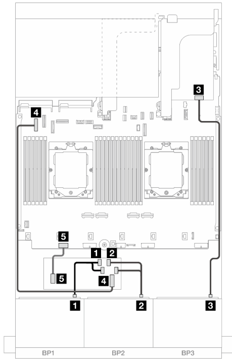
図 461. 2つのプロセッサが取り付けられた場合のケーブル配線
