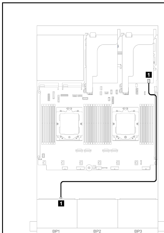
図 433. SAS/SATA ケーブル配線
