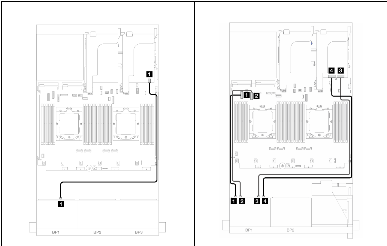
図 372. SAS/SATA ケーブル配線
