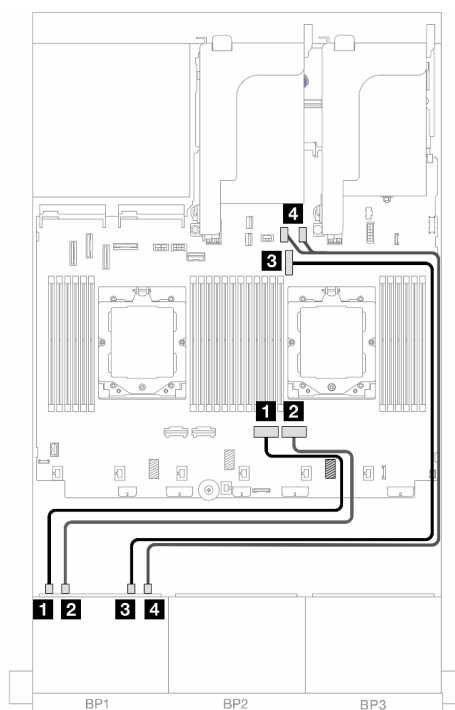
図 385. 1つのプロセッサが取り付けられた場合のケーブル配線
