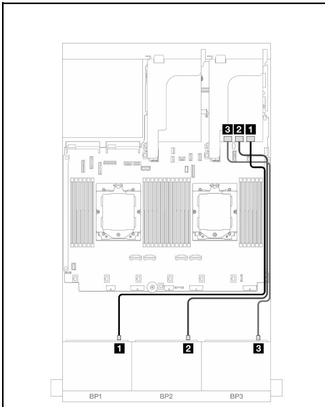
図 457. 前面バックプレーンのケーブル配線
