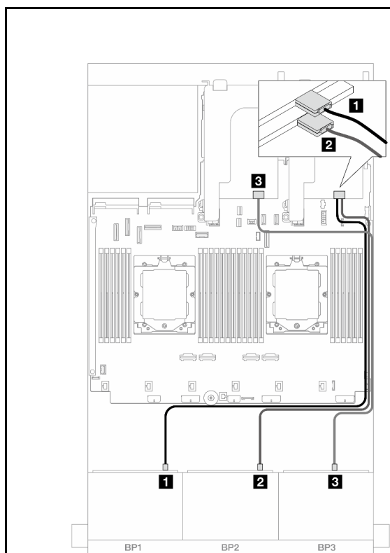
図 506. SAS/SATA ケーブル配線
