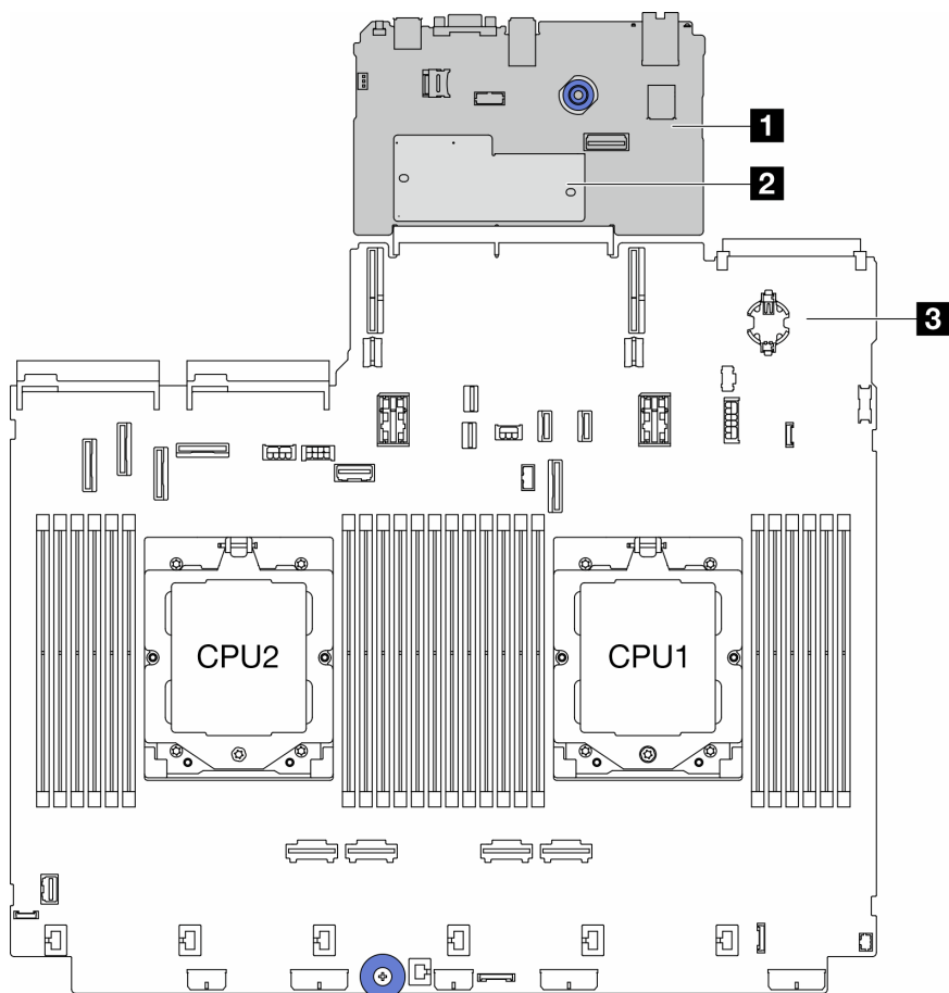
図 11. システム・ボード・アセンブリーのレイアウト
