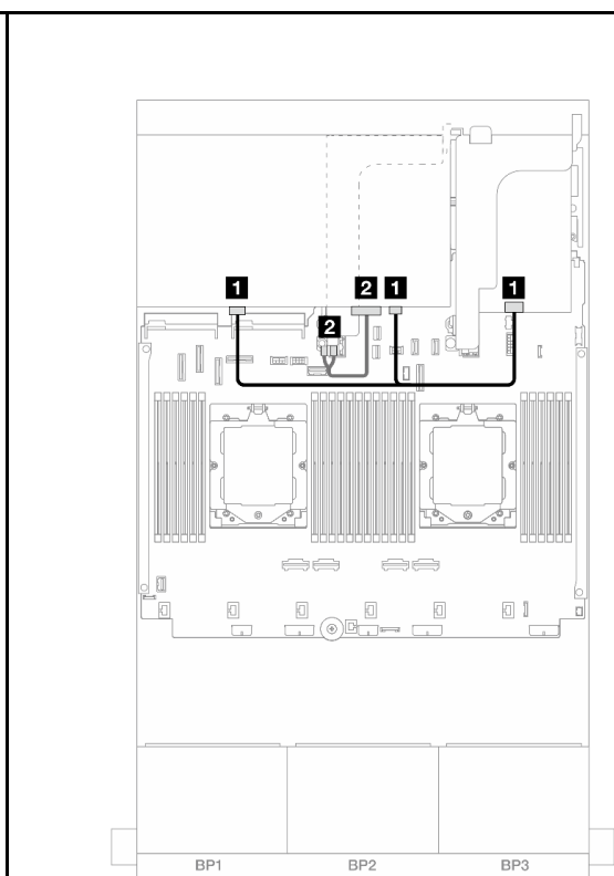
図 460. 背面バックプレーンのケーブル配線
