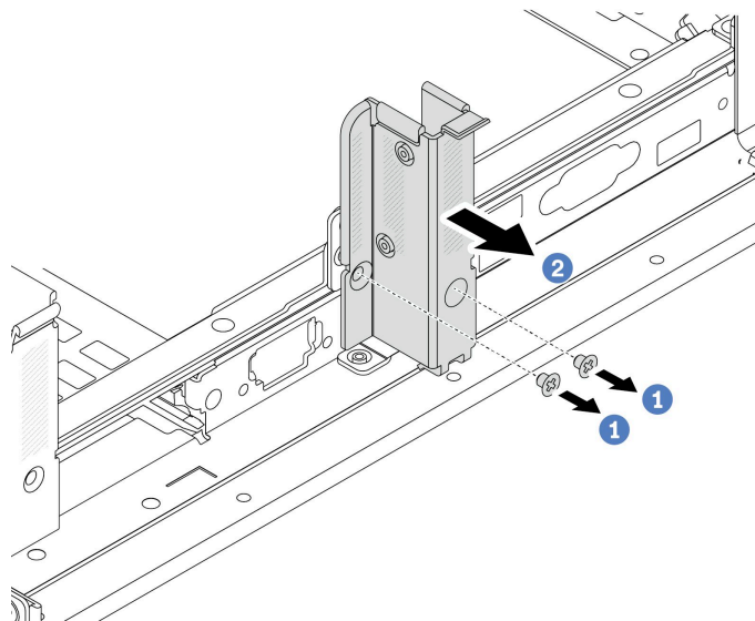
図 227. B1 背面壁ブラケットの取り外し (中央)
