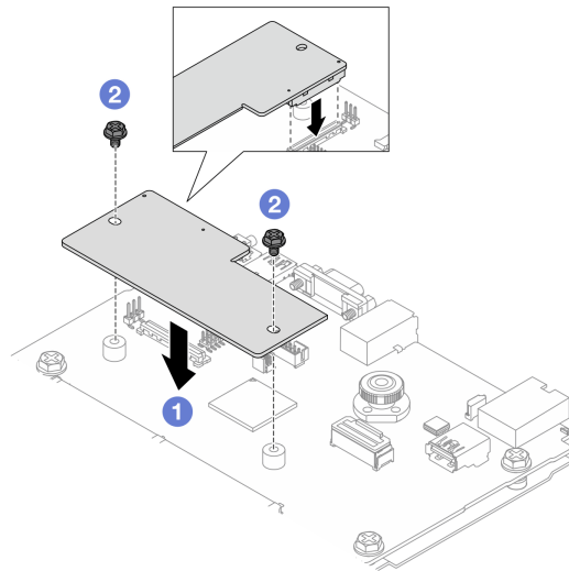
図 291. ファームウェアおよび RoT セキュリティー・モジュールの取り付け
