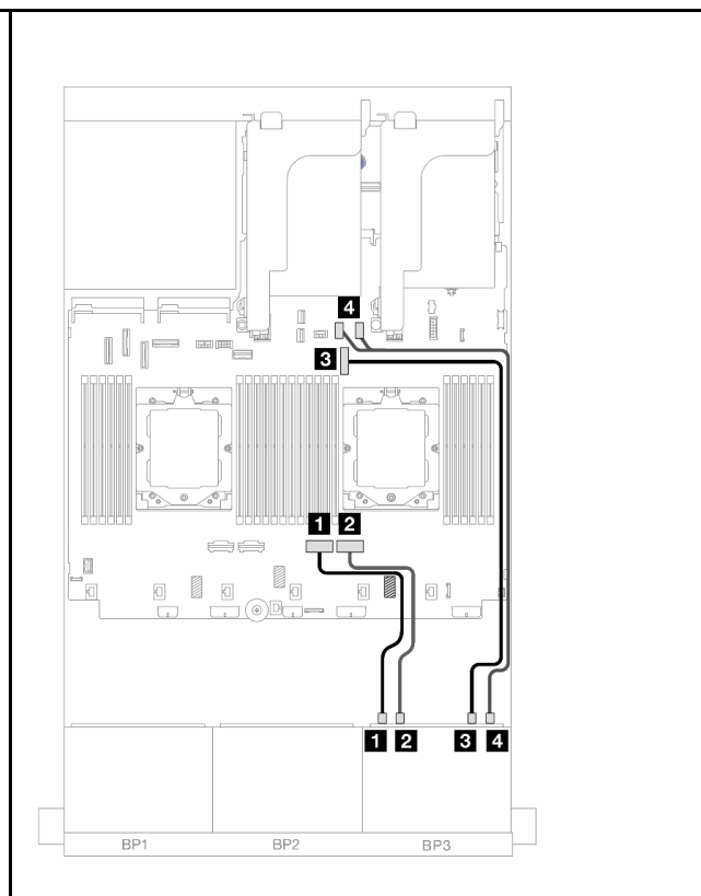
図 523. NVMe ケーブル配線
