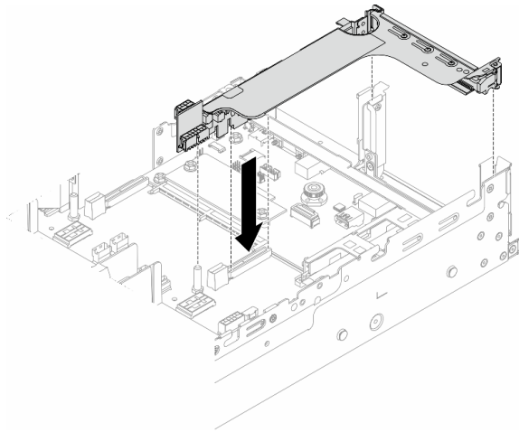
図 308. ライザー・アセンブリーの取り付け
