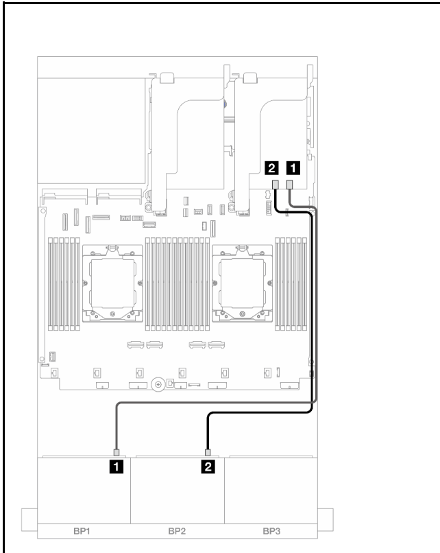
図 526. SAS/SATA ケーブル配線
