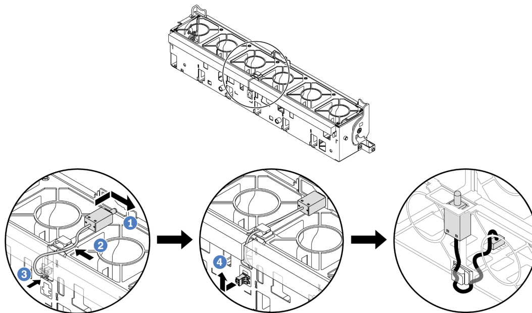
図 100. 侵入検出スイッチの取り付け
