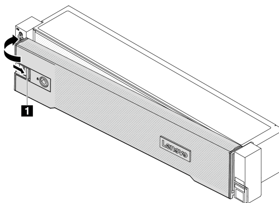
図 287. セキュリティー・ベゼルの取り付け
