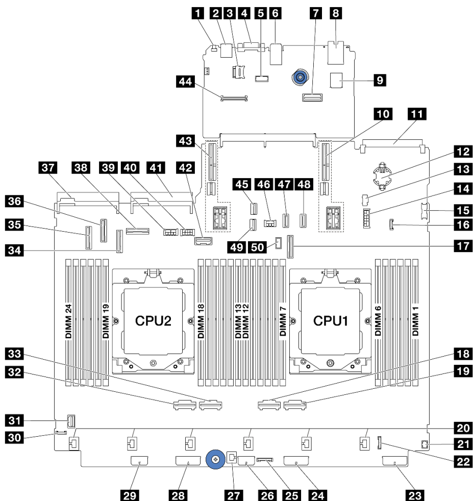
図 12. システム・ボード・アセンブリー・コネクタ
