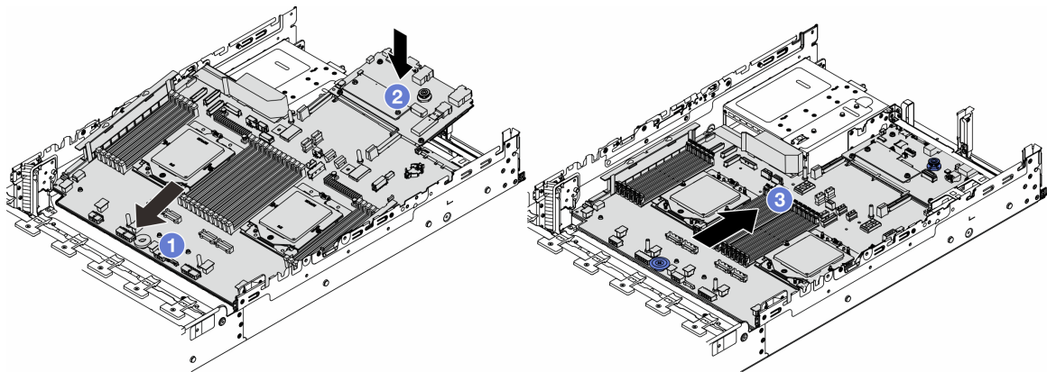
図 297. システム・ボード・アセンブリーの取り付け
