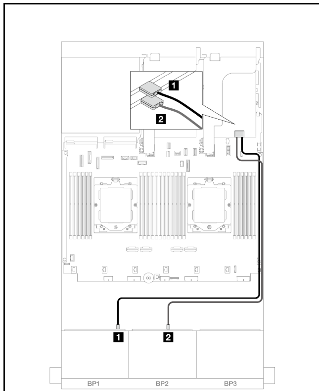
図 414. SAS/SATA ケーブル配線
