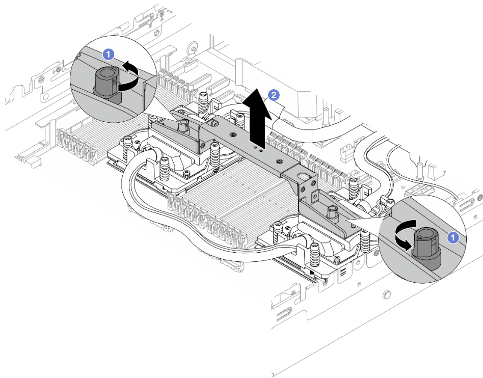
図108. モジュール・ハンドルの取り外し
