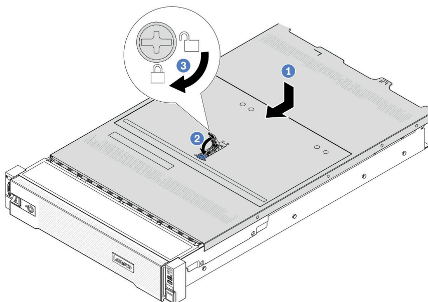
図 310. トップ・カバーの取り付け
