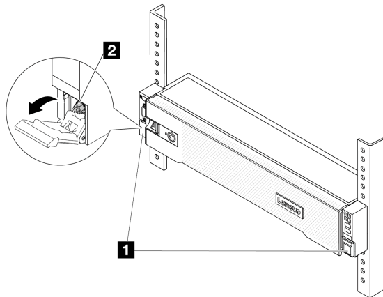
図20. ラックからのサーバーを取り外す
