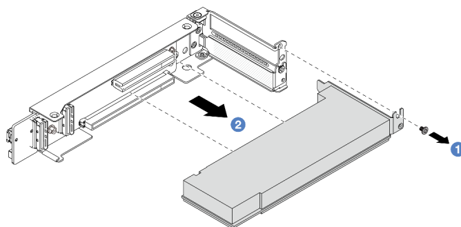
図270. 4LP ライザー 3/4 アセンブリーからの PCIe アダプターの取り外し
