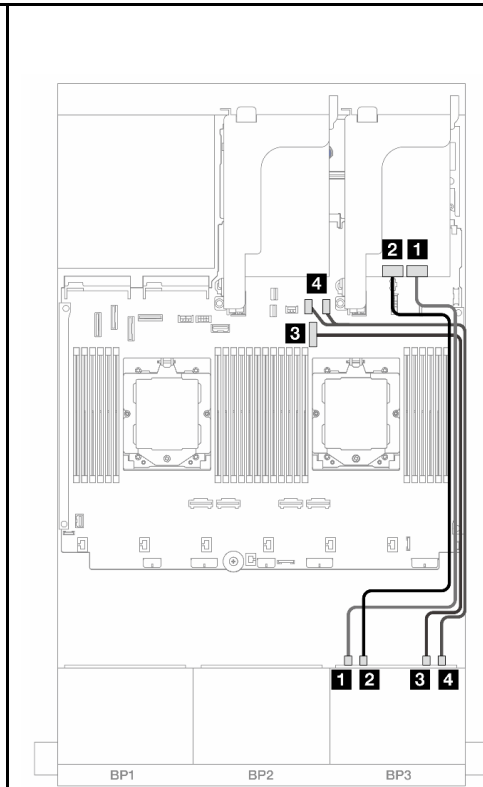
図 529. NVMe ケーブル配線
