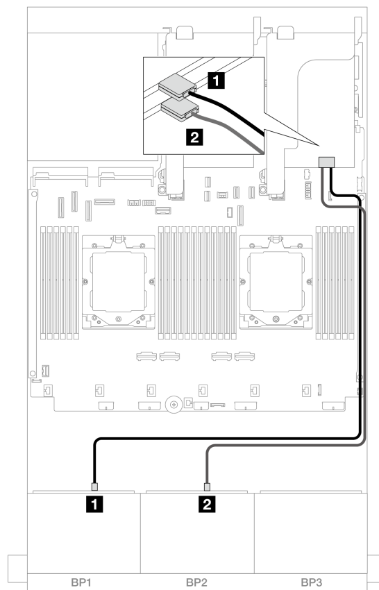
図 402. トライモード 8i アダプターへの信号ケーブル配線
