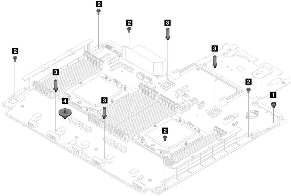
図 600. プロセッサ・ボードからのねじの取り外し
