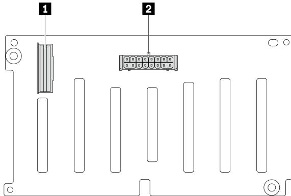
図 311. 8 個の 2.5 型 SAS/SATA バックプレーン・コネクタ
