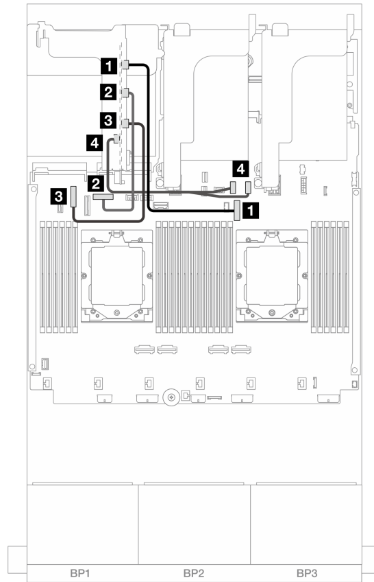
図 349. x16/x16 Gen 4 PCIe ライザー・カード 3 向け信号ケーブル接続
