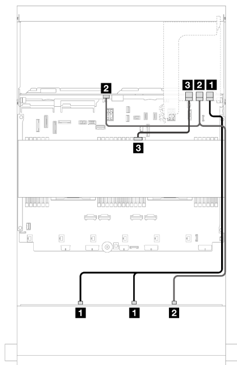
図 565. 前面/背面バックプレーン信号ケーブルの配線
