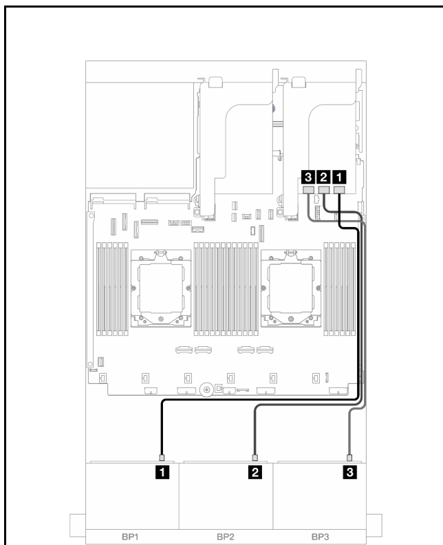
図 469. 前面バックプレーンのケーブル配線
