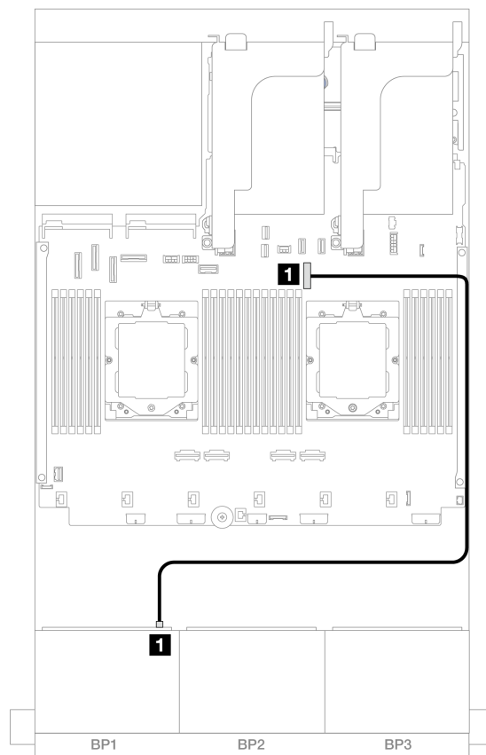
図374. オンボード・コネクタへの SAS/SATA ケーブル配線
