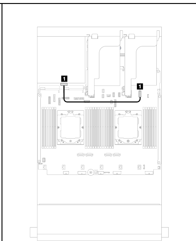
図 554. 背面バックプレーン電源ケーブルの配線
