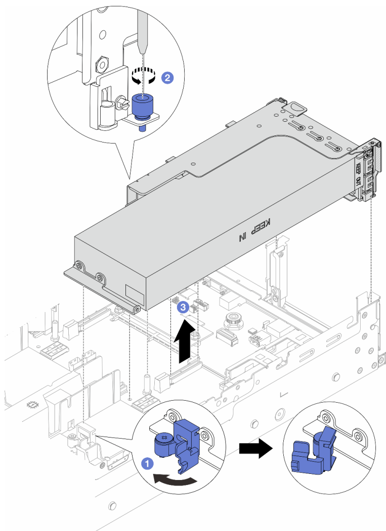
図 88. ライザー 1 アセンブリーへの GPU アダプターの取り外し
