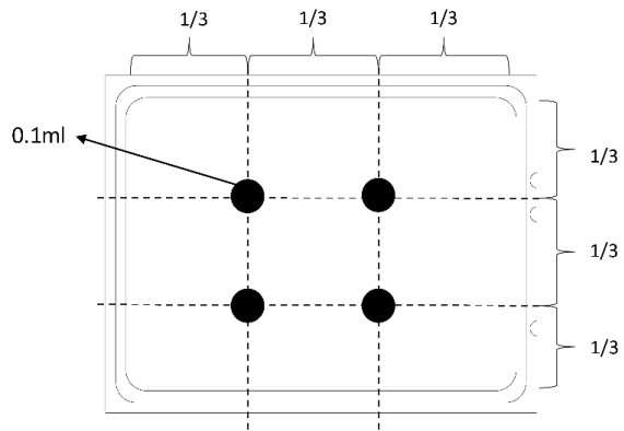
図 200. 熱伝導グリースの塗布
