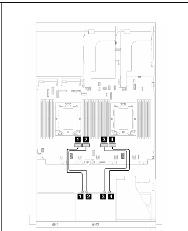
図 415. NVMe ケーブル配線
