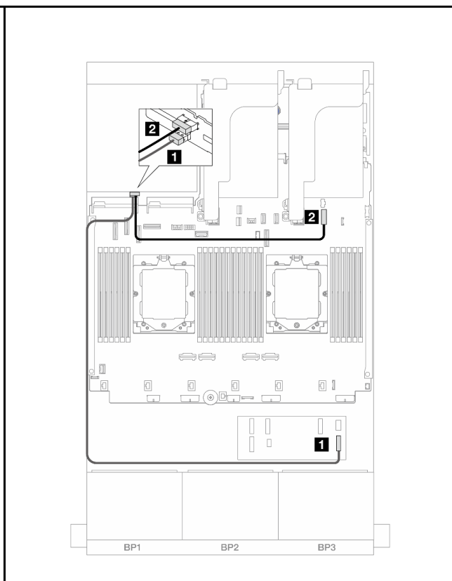
図 443. 背面バックプレーンのケーブル配線
