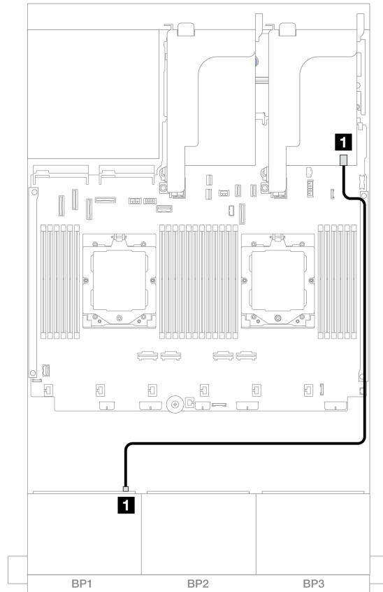
図 426. 8i アダプターへの SAS/SATA ケーブル配線
