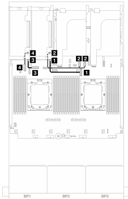
図354. ライザー・カード 3/4 信号ケーブル配線
