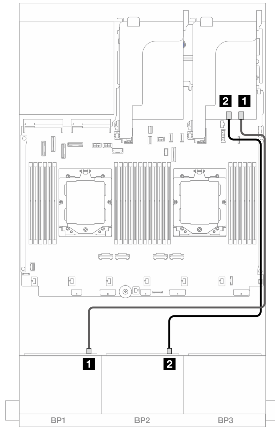
図 517. 16i RAID/HBA アダプターへの SAS/SATA ケーブル配線
