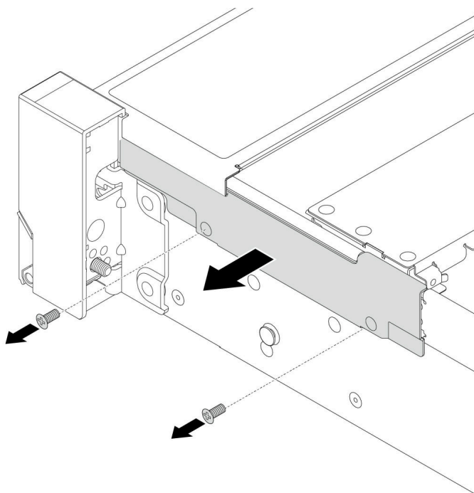
図 204. ケーブル保持具の取り外し
