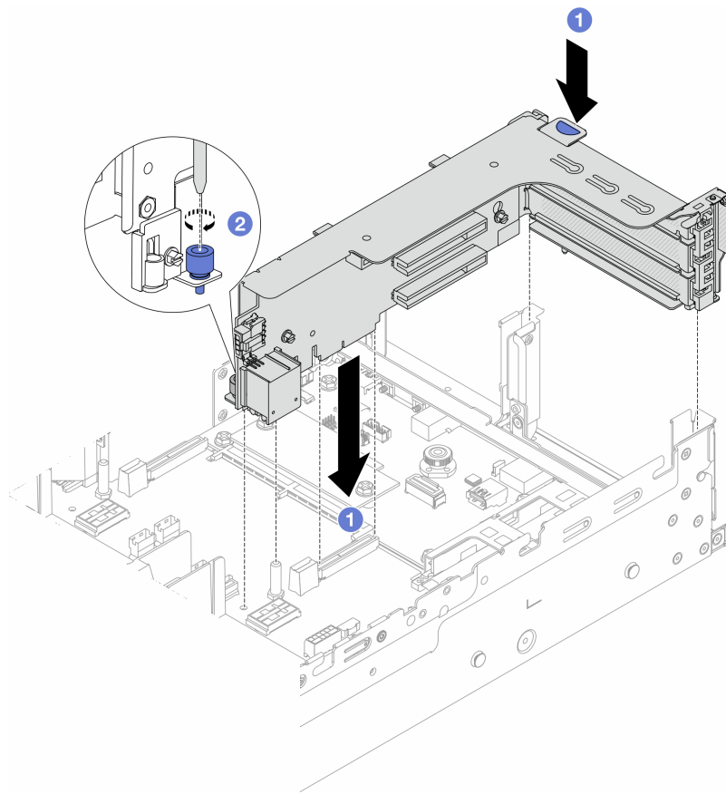
図280. ライザー 1 アセンブリーの取り付け
