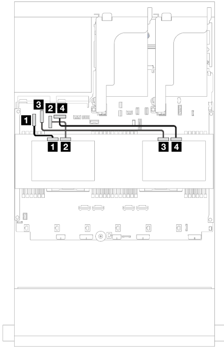
図 561. 中央バックプレーン信号ケーブル配線
