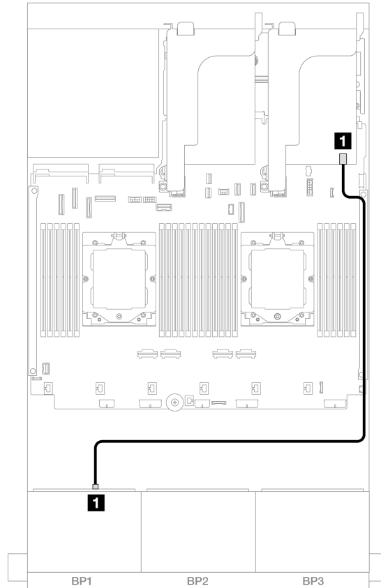
図 495. 8i アダプターへの SAS/SATA ケーブル配線
