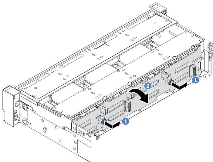
図 75. 3.5 型ドライブ・バックプレーンの取り外し
