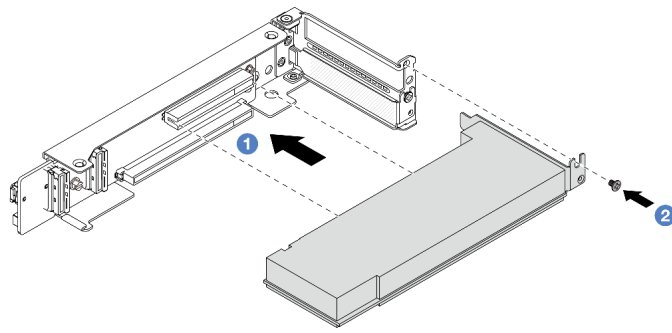
図 279. PCIe アダプターの 4LP ライザー 3/4 アセンブリーへの取り付け
