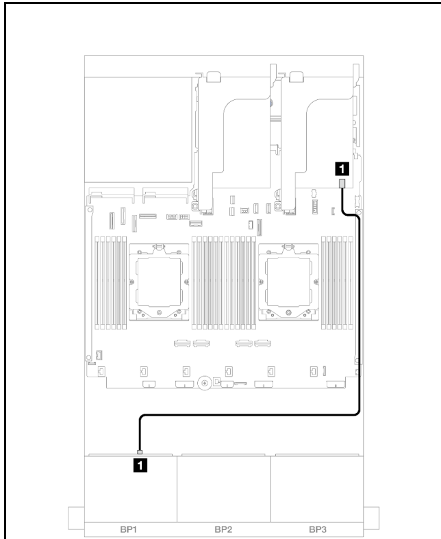
図 382. SAS/SATA ケーブル配線
