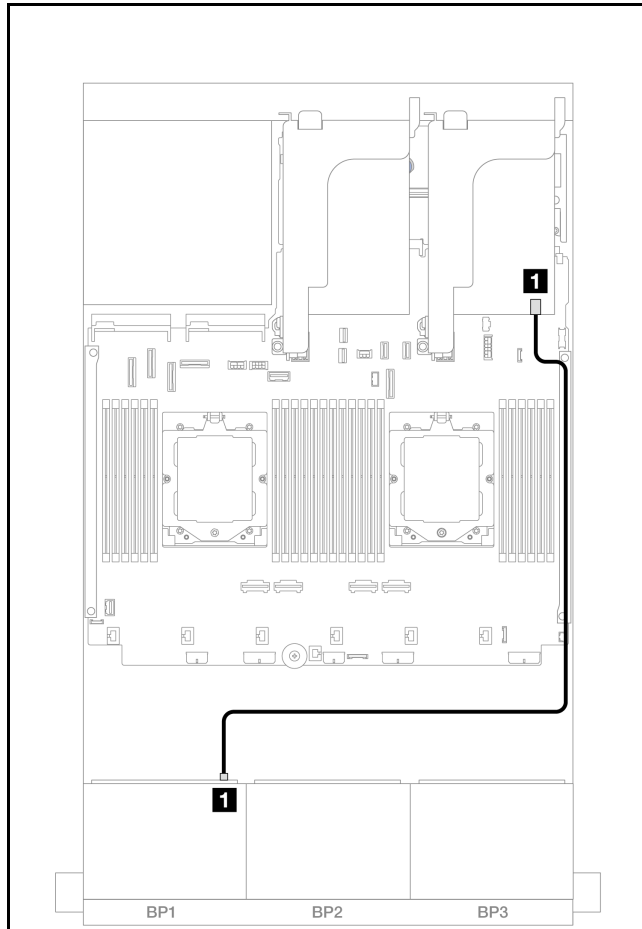
図 501. SAS/SATA ケーブル配線
