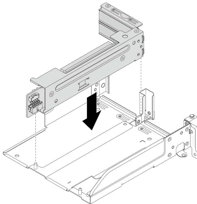
図 283. ライザー 3/4 アセンブリの取り付け
