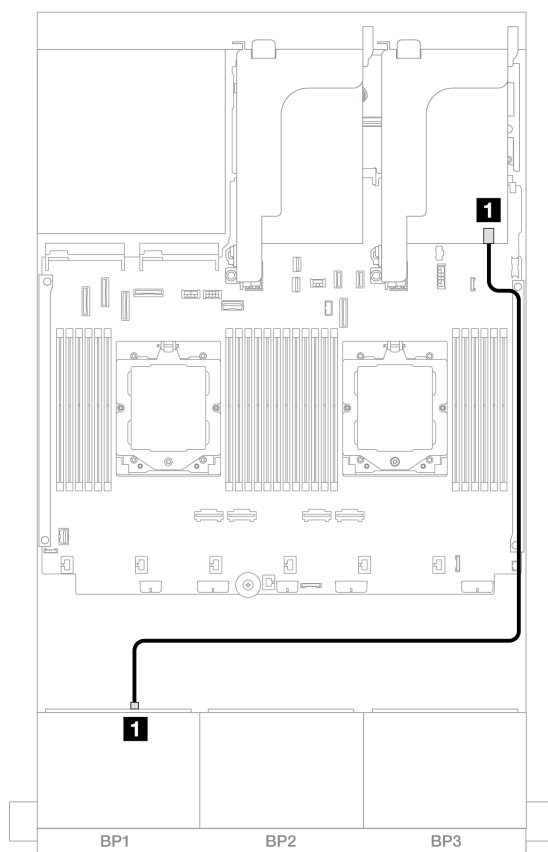
図 365. 8i/16i RAID/HBA アダプターへの SAS/SATA ケーブル配線
