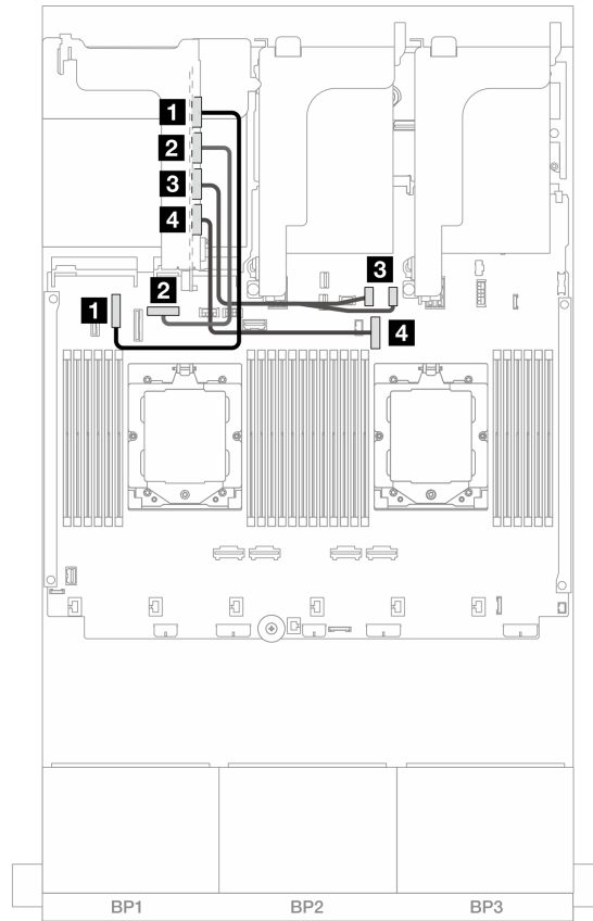
図 352. x16/x16 Gen 5 PCIe ライザー・カード 3 向け信号ケーブル接続
