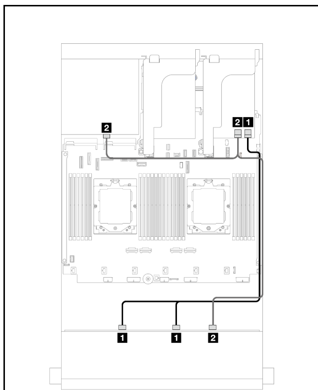
図 553. 前面/背面バックプレーン信号ケーブルの配線
