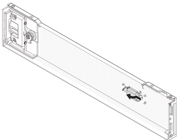
図 286. キーの取り外し
