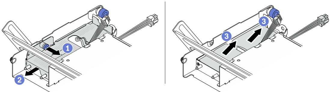
図 222. 中央ドライブ・ケージからの RAID フラッシュ電源モジュールの取り外し
