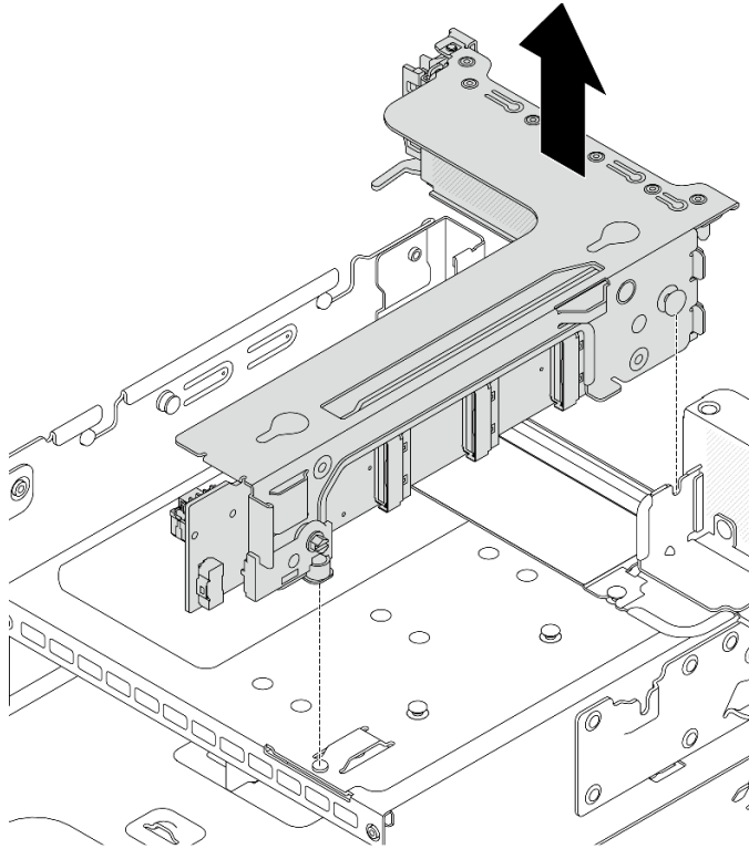
図 265. ライザー・アセンブリー 3 の取り外し
