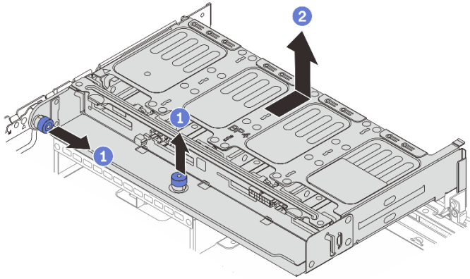
図 247. 8 x 2.5 型背面ドライブ・ケージの取り外し
