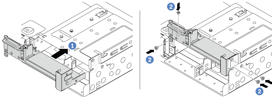
図 231. 左側 C1 背面壁ブラケットの取り付け (右)
