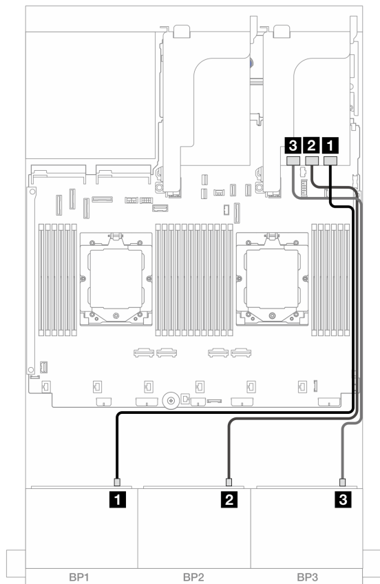
図 437. 32i アダプターへの SAS/SATA ケーブル配線
