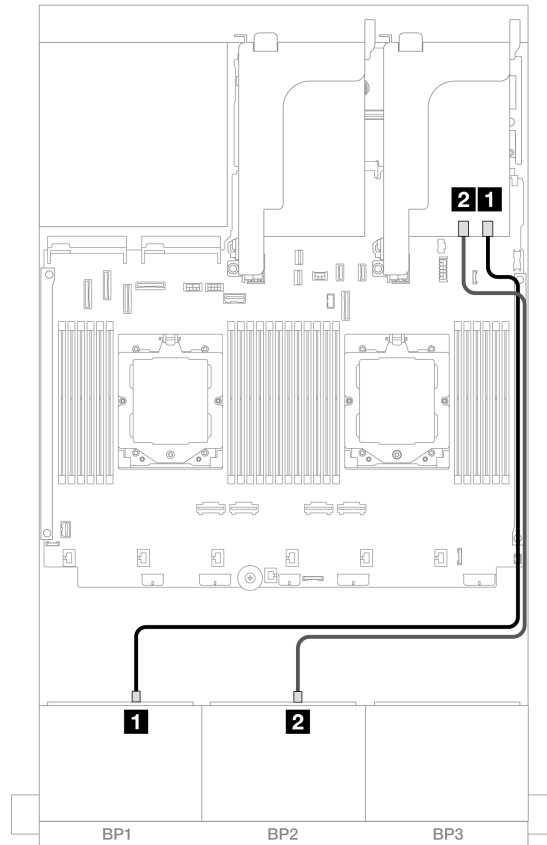
図 403. トライモード 16i アダプターへの信号ケーブル配線
