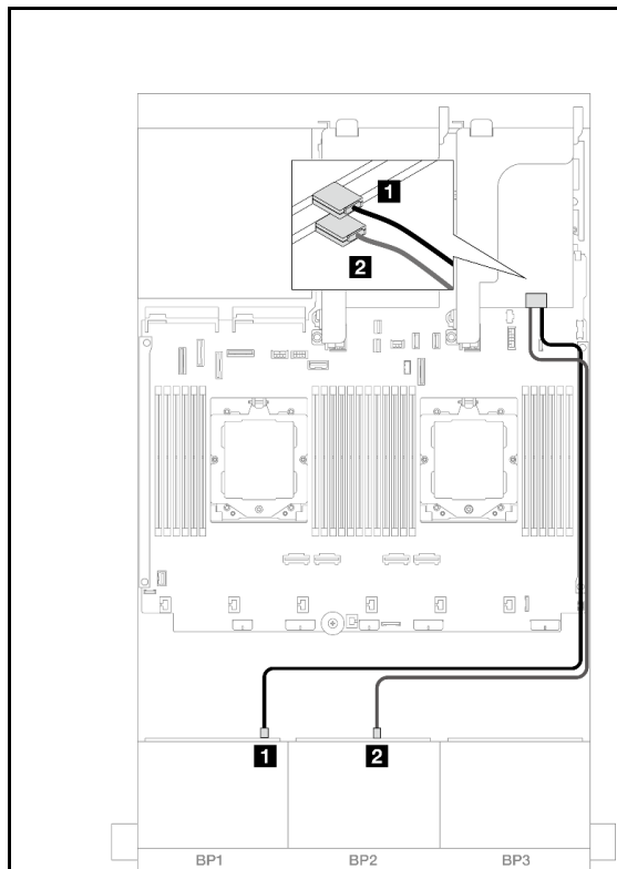
図 418. SAS/SATA ケーブル配線
