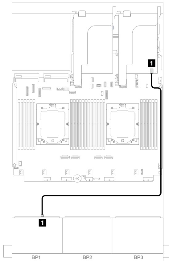
図 377. 8i RAID/HBA アダプターへの SAS/SATA ケーブル配線
