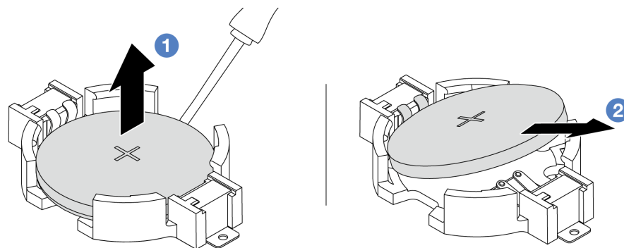
図 36. CMOS バッテリーの取り外し
