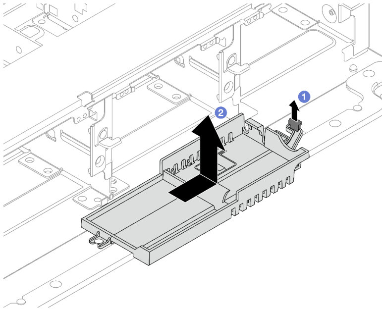
図215. スーパーキャップ・ホルダーの取り外し
