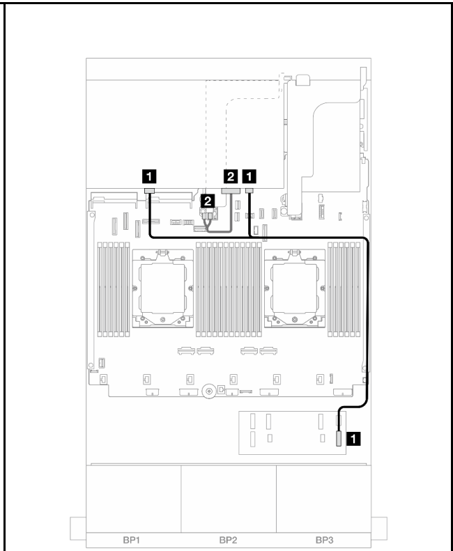
図 465. 背面バックプレーンのケーブル配線
