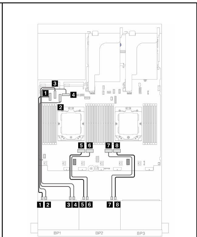
図 434. NVMe ケーブル配線
