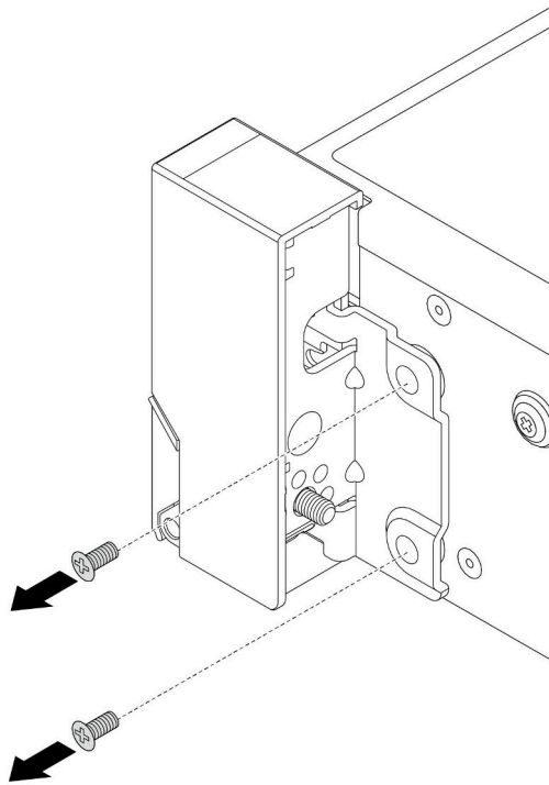
図 205. ねじの取り外し
