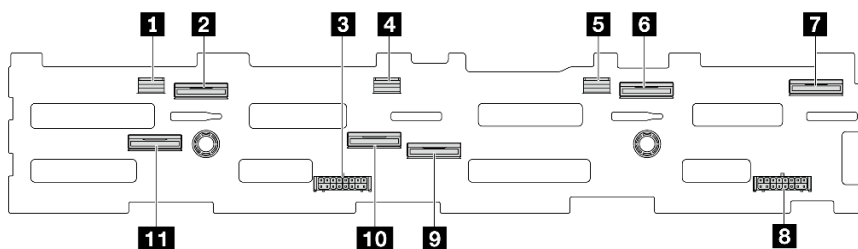
図 317. 12 x 3.5 型 AnyBay バックプレーン・コネクタ
