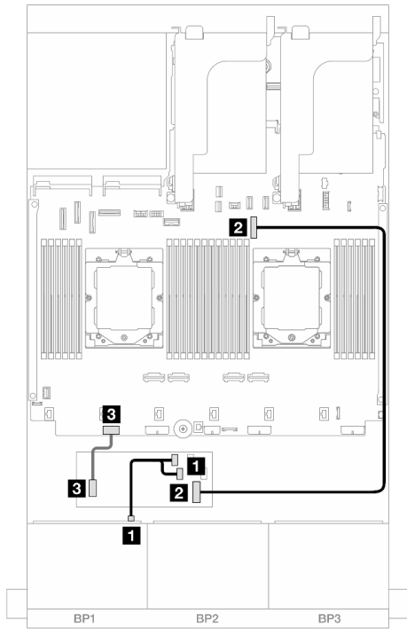
図 368. SAS/SATA ケーブル配線
