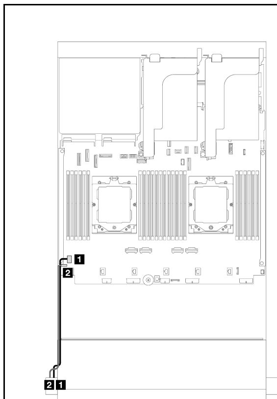
図 330. VGA コネクタおよび外部診断コネクタ (左のラック・ラッチ)
