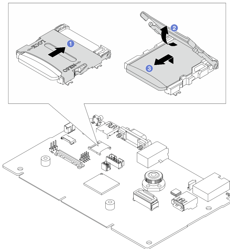
図 181. MicroSD カードの取り外し
