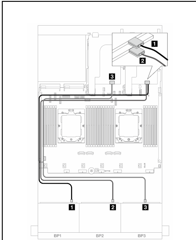
図 512. SAS/SATA ケーブル配線
