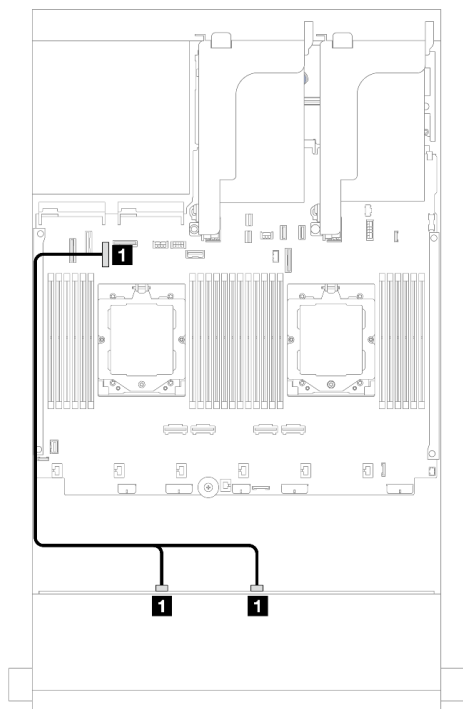
図 571. SAS/SATA ケーブル配線
