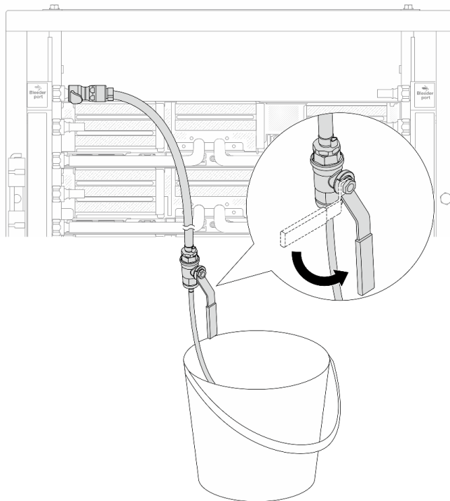
図 173. 供給側のブリーダのバルブを開く
