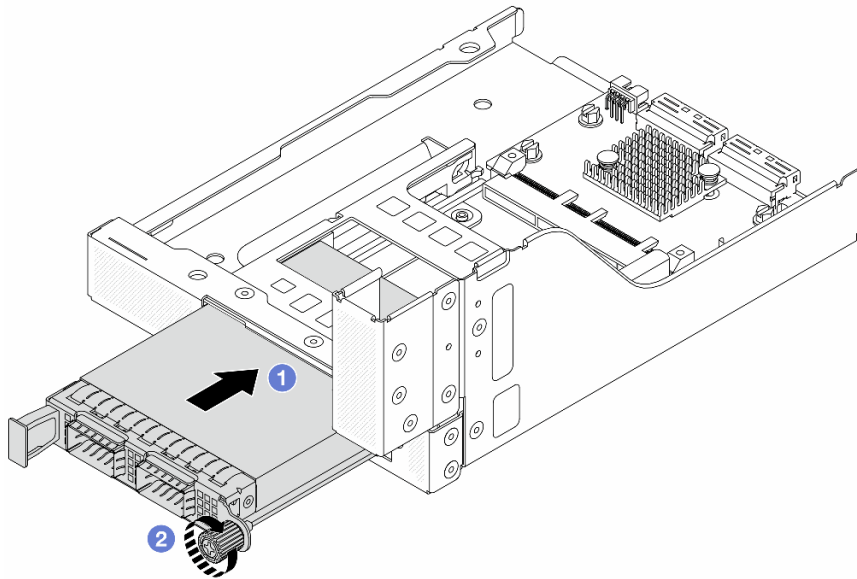
図 57. OCP モジュールの取り付け
