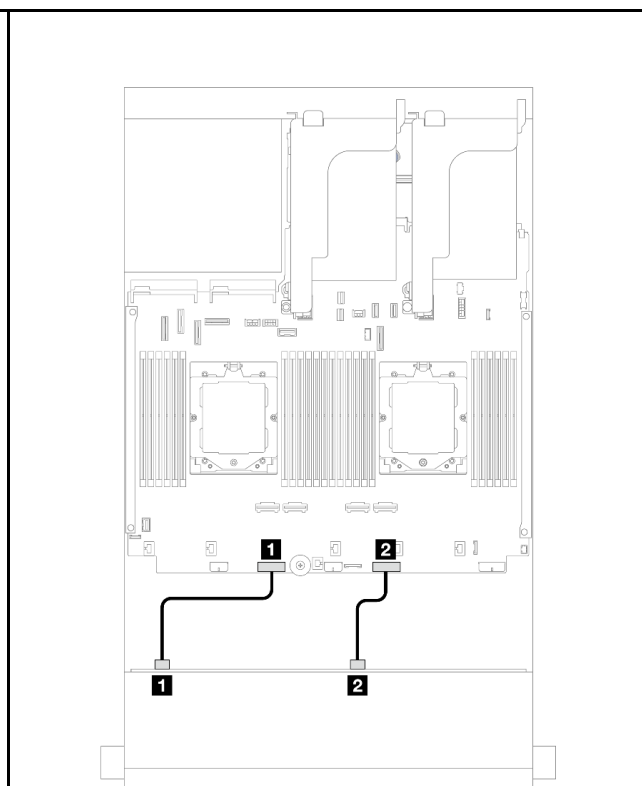
図 541. 12 x 3.5 型 SAS/SATA/AnyBay バックプレーン用電源ケーブル接続
