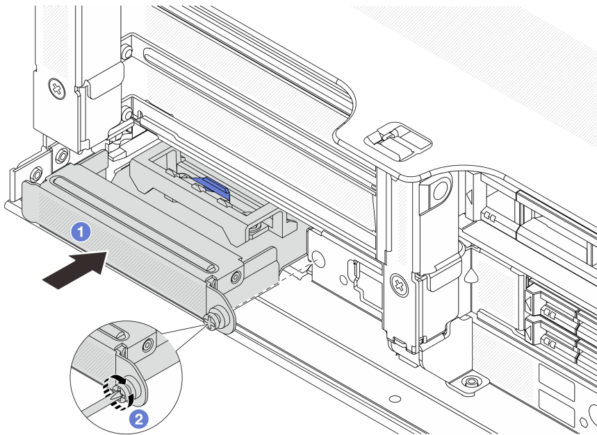
図 61. 背面 OCP 変換コネクタ・カードの取り付け
