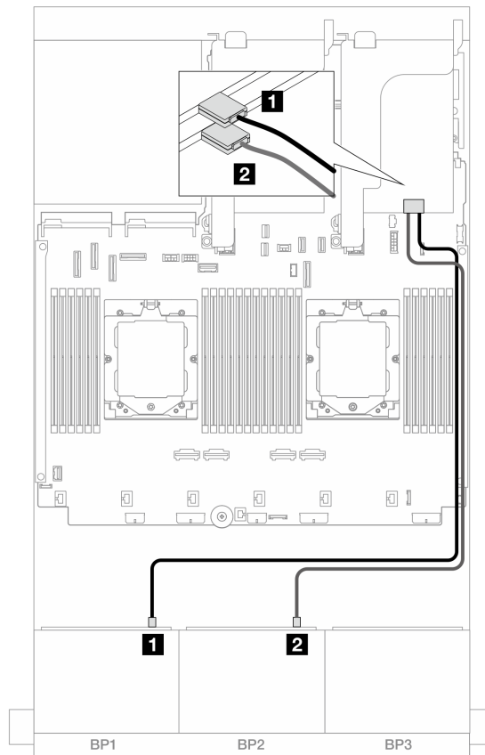
図 514. 8i アダプターへの SAS/SATA ケーブル配線
