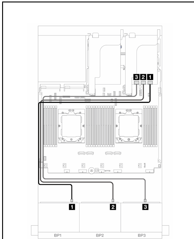
図510. SAS/SATA ケーブル配線
