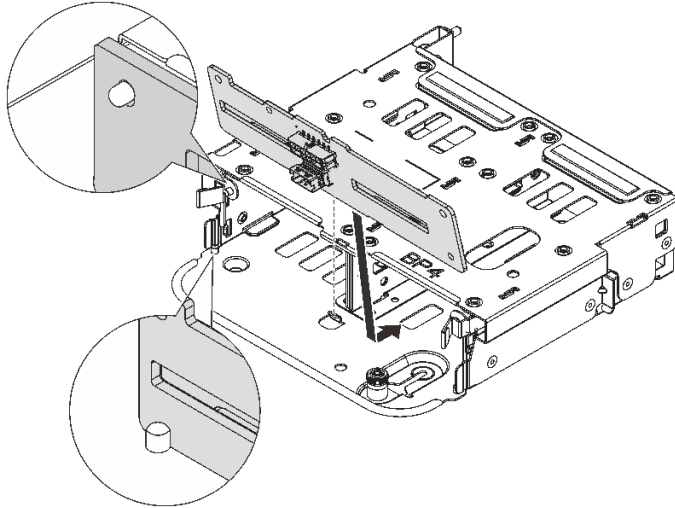
図 245. 4 x 2.5 型背面ドライブ・バックプレーンの取り付け
