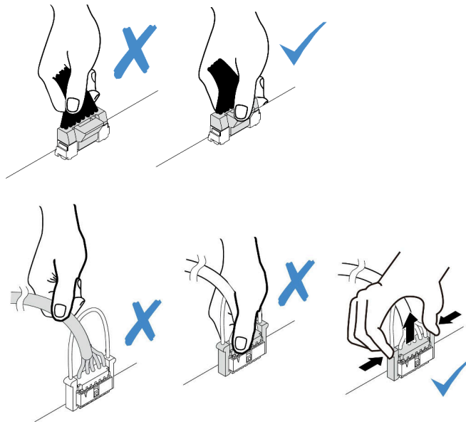
図95. ケーブルのシステム・ボード・アセンブリーからの切り離し
