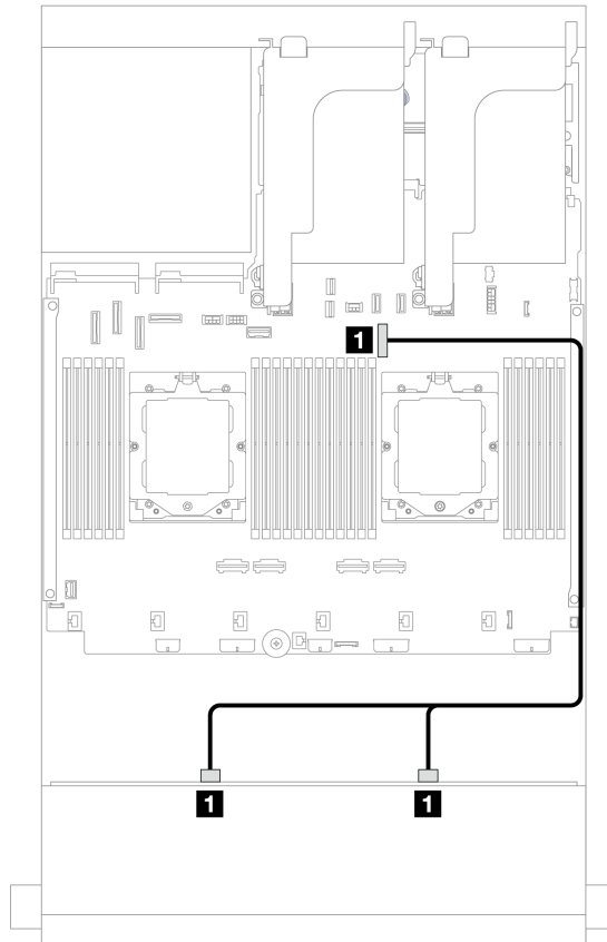
図 542. オンボード SATA コネクタのケーブル配線
