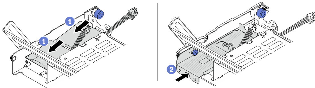
図 223. 中央ドライブ・ケージへの RAID フラッシュ電源モジュールの取り付け
