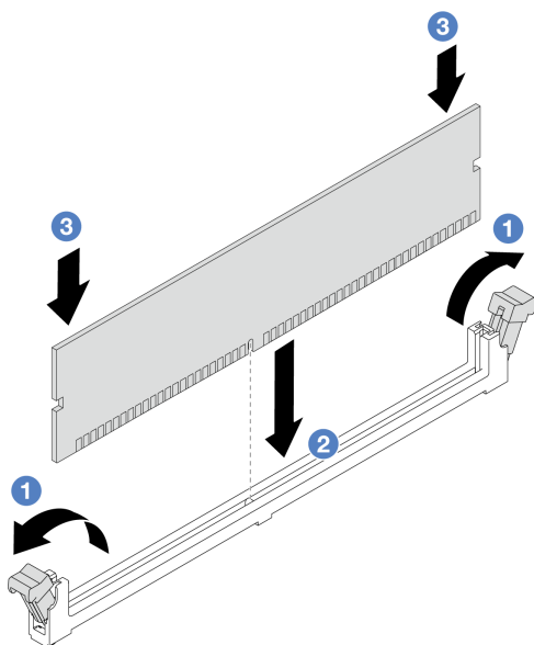
図 180. メモリー・モジュールの取り付け
