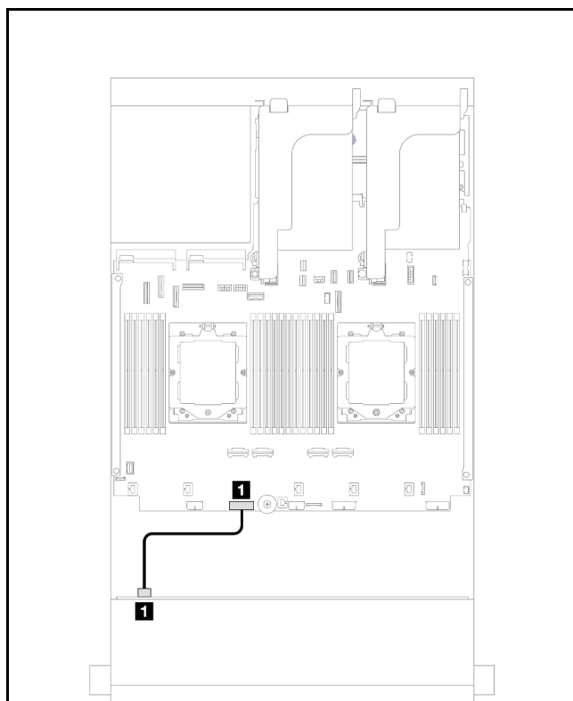
図 540. 8 x 3.5 型 SAS/SATA バックプレーンおよび 12 x 3.5 型 SAS/SATA エクスパンダー・バックプレーン用電源ケーブル接続
