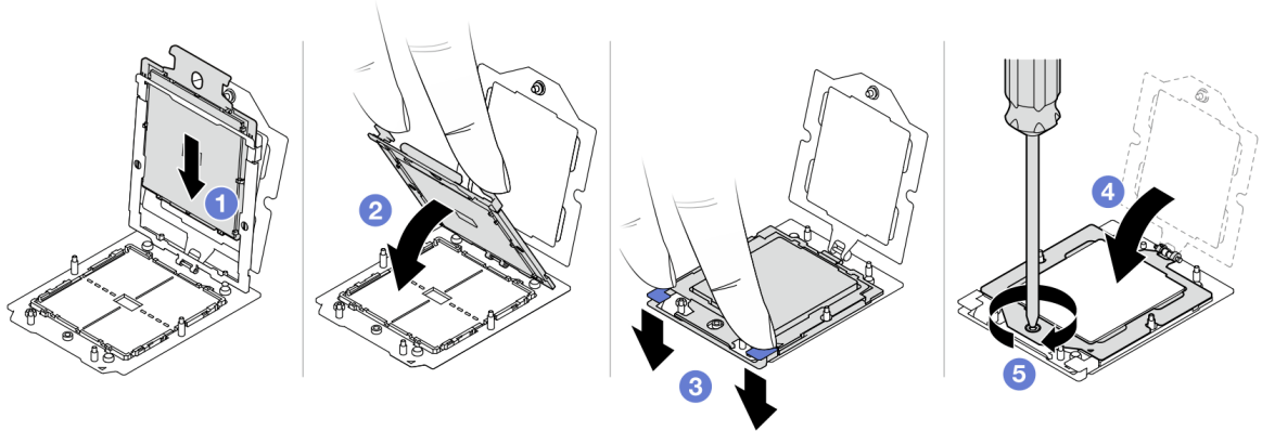
図 199. プロセッサの取り付け
