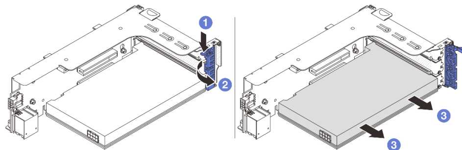
図 268. ライザー 1 または 2 アセンブリーからの PCIe アダプターの取り外し
