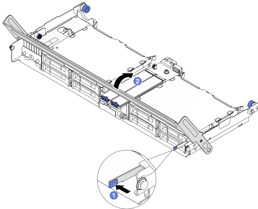
図 126. 中央ドライブ・ケージのハンドルを閉じる
