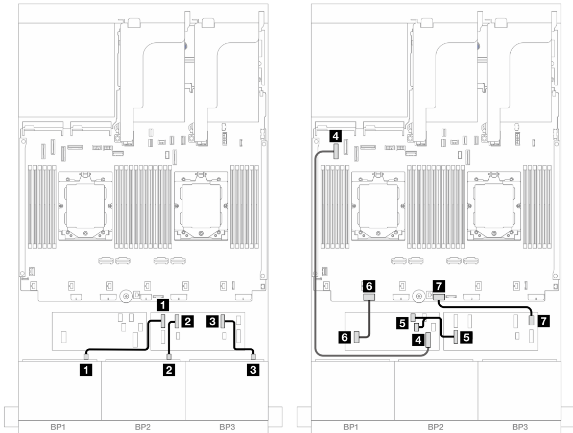
図 466. CFF エクスパンダーおよび CFF 16i アダプターへの SAS/SATA ケーブル配線
