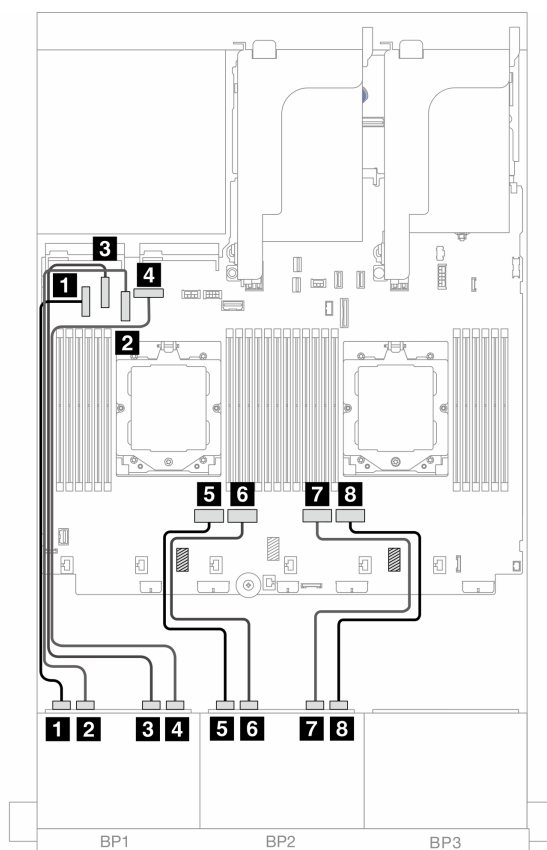
図 404. オンボード PCIe コネクタへの NVMe ケーブル配線
