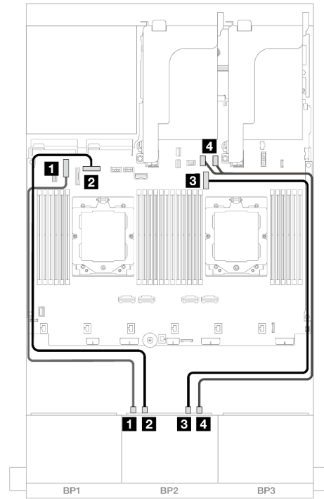
図 413. NVMe ケーブル配線
