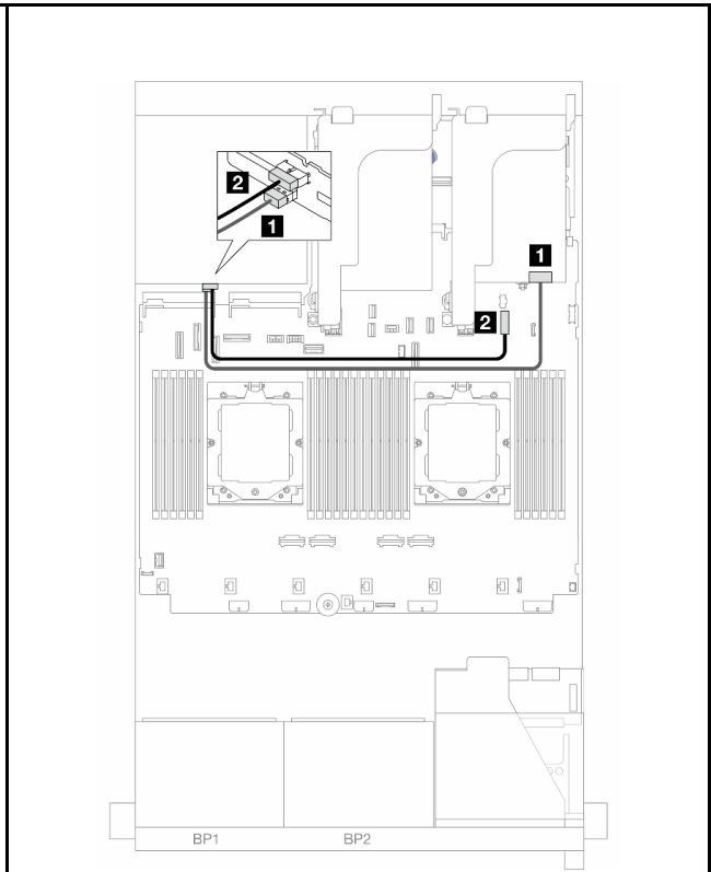
図 394. 背面バックプレーンのケーブル配線
