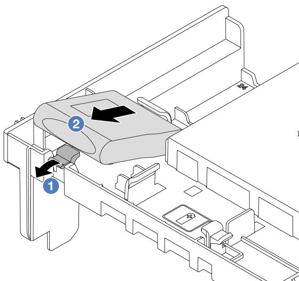
図218. エアー・バッフルからの RAID フラッシュ電源モジュールの取り外し
