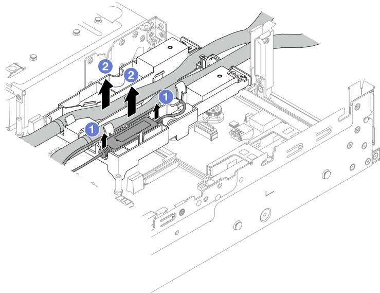
図103. ホースとモジュールの取り外し
