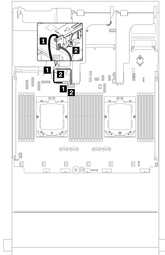
図 346. ライザー・カード 3 電源および側波帯接続
