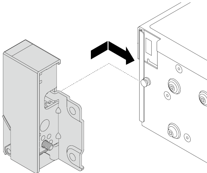
図 207. ラック・ラッチの取り付け
