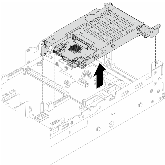
図 233. 7mm SSD ライザー・ケージの取り外し
