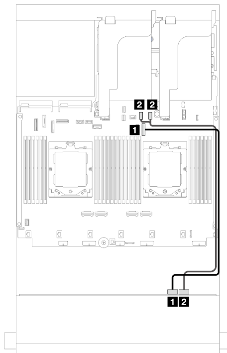
図 572. NVMe ケーブル配線
