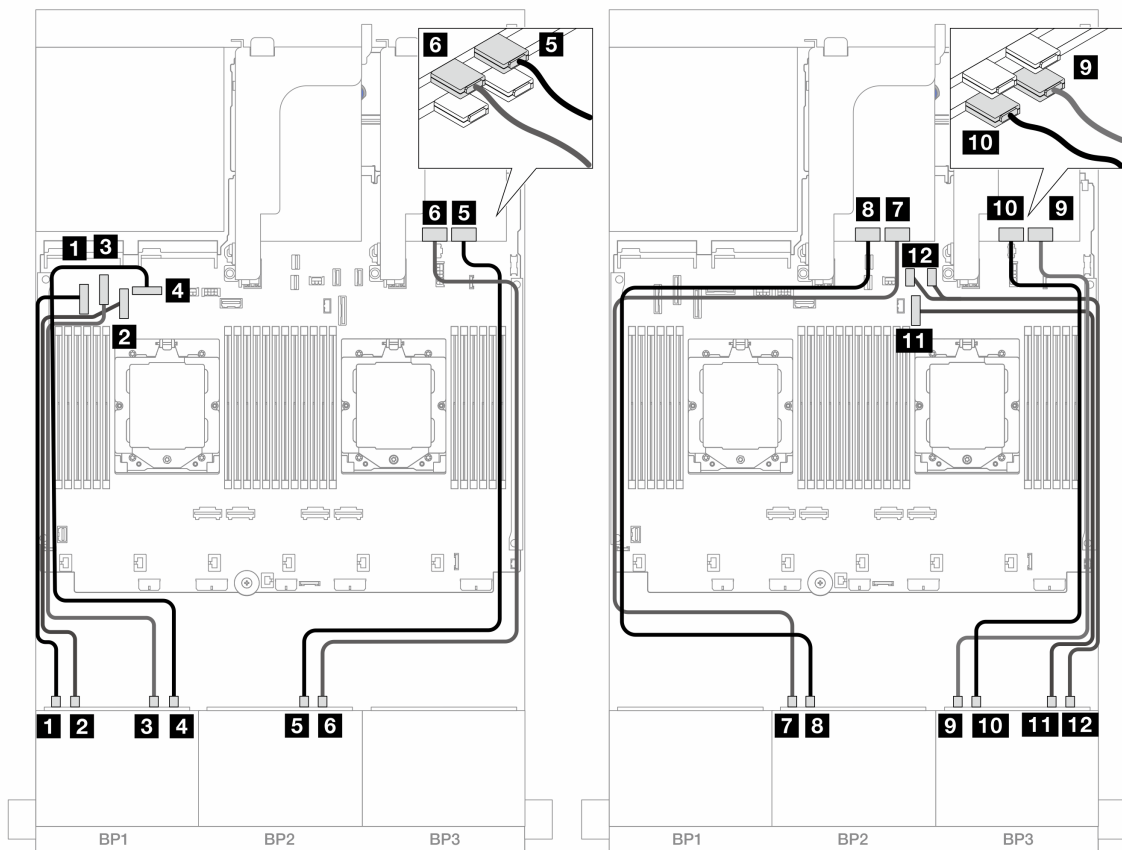
図 492. オンボード・コネクタおよびリタイマー・カードへの NVMe ケーブル配線
