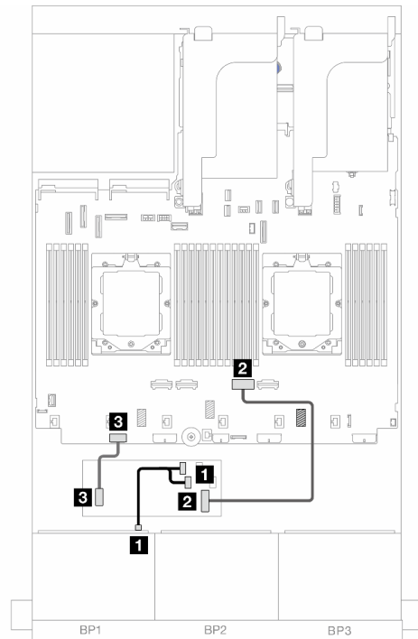
図364. 1つのプロセッサが取り付けられた場合のケーブル配線
