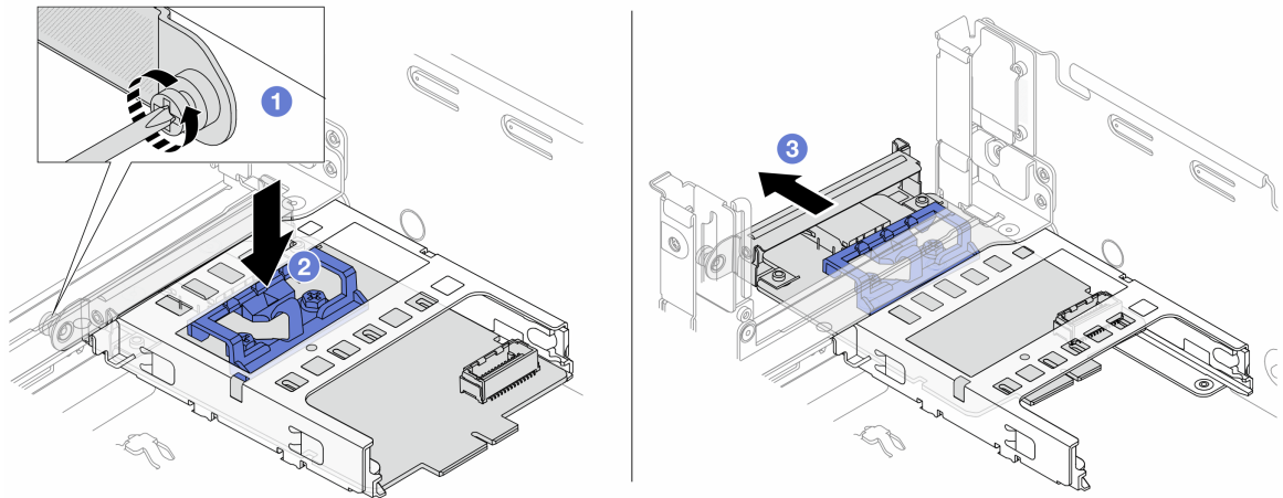
図 130. 管理 NIC アダプターの取り外し
