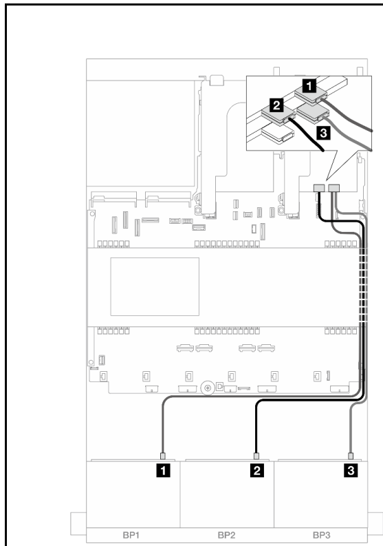
図 471. 前面バックプレーンのケーブル配線
