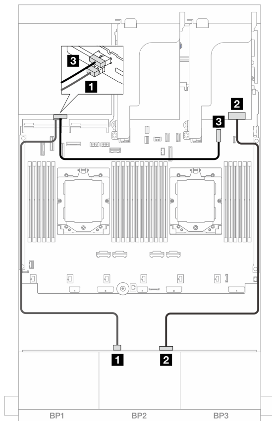
図 533. 前面/背面バックプレーンのケーブル配線
