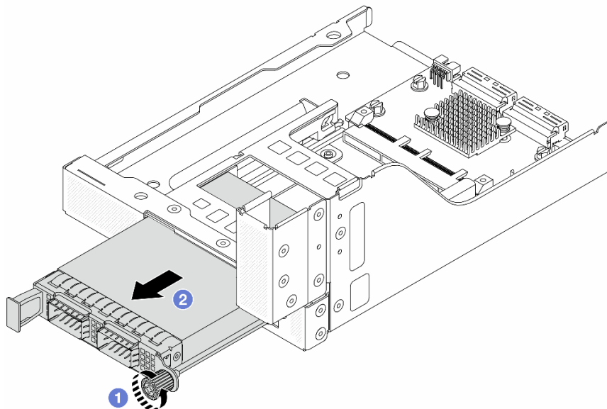
図 42. OCP モジュールの取り外し
