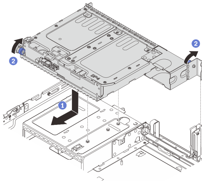
図 254. 2 x 3.5 型背面ドライブ・ケージの取り付け
