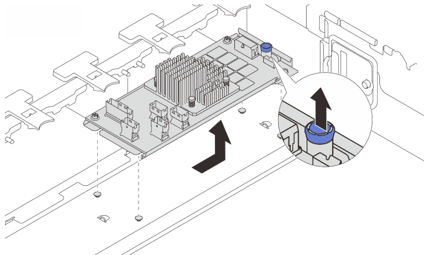
図96. 内蔵 CFF アダプターの取り外し
