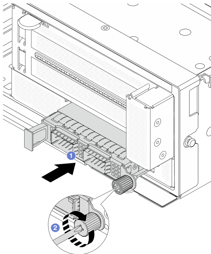
図 51. 前面 OCP モジュールの取り付け
