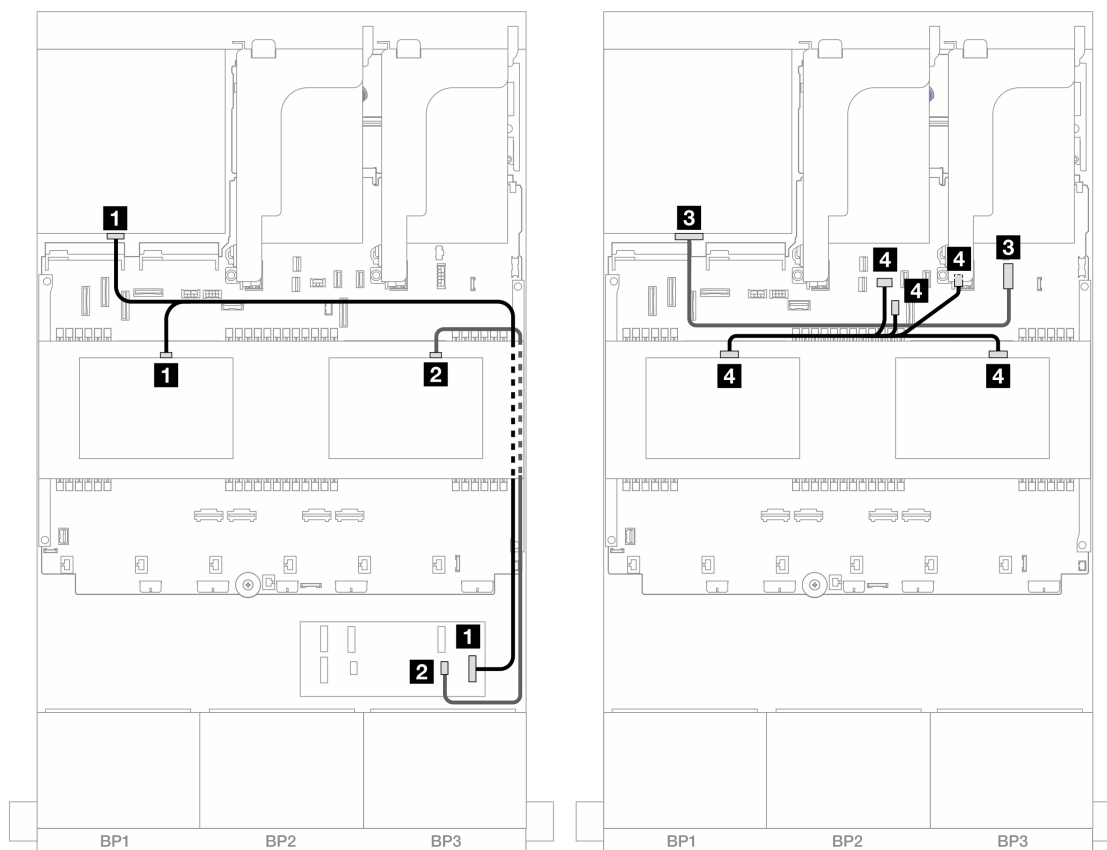
図 480. 中央/背面バックプレーンのケーブル配線
