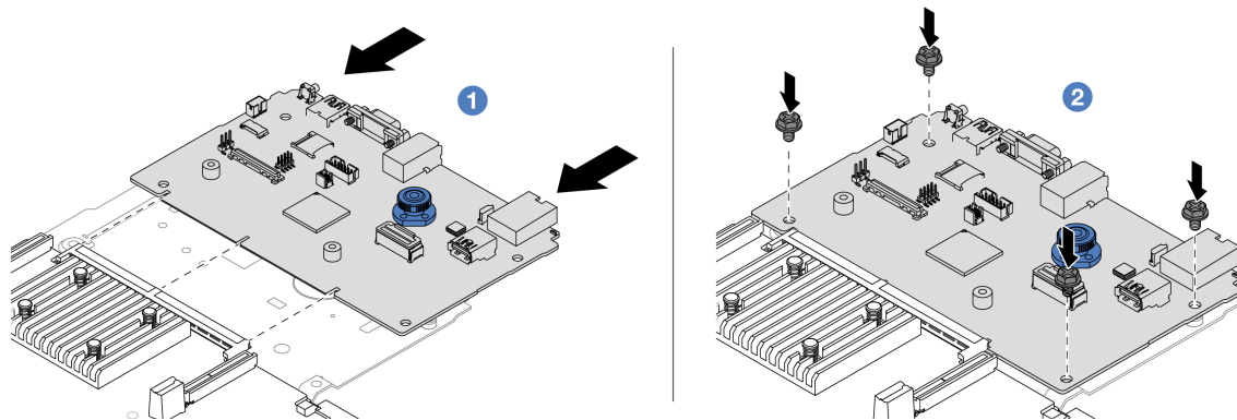
図296. プロセッサ・ボードへのシステム I/O ボードの取り付け
