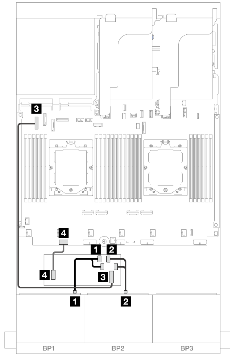
図 412. SAS/SATA ケーブル配線
