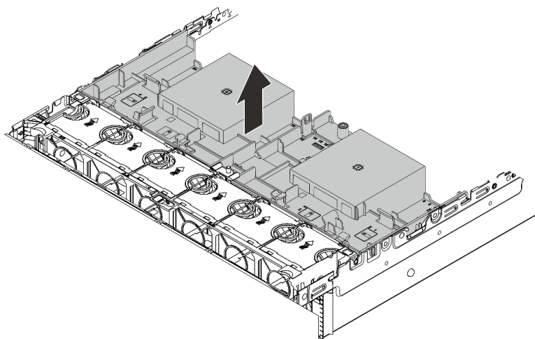
図 30. エアー・バッフルの取り外し
