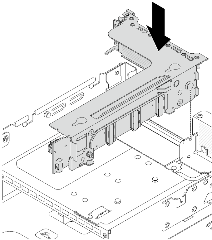
図281. ライザー 3 アセンブリーの取り付け
