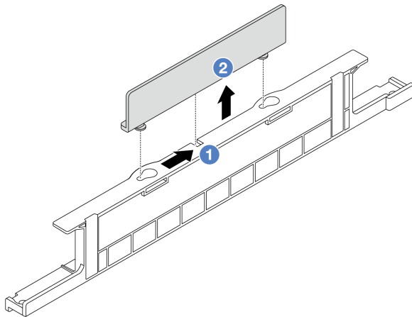
図 34. 2U ケーブル壁ブラケットの取り外し
