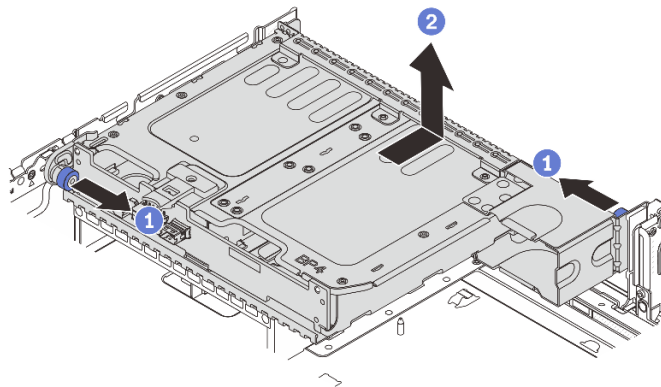
図 251. 2 x 3.5 型背面ドライブ・ケージの取り外し
