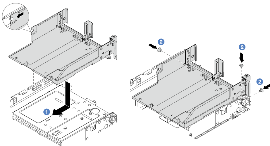
図282. ライザー・ケージ・トレイの取り付け
