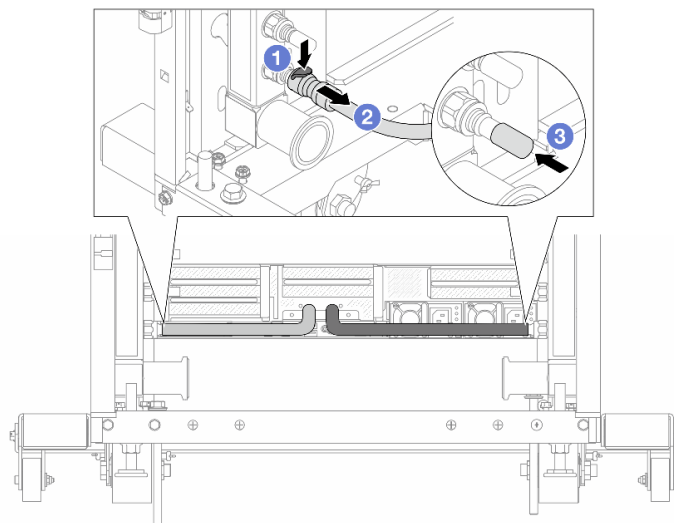
図161. クイック・コネクト・プラグの取り外し
