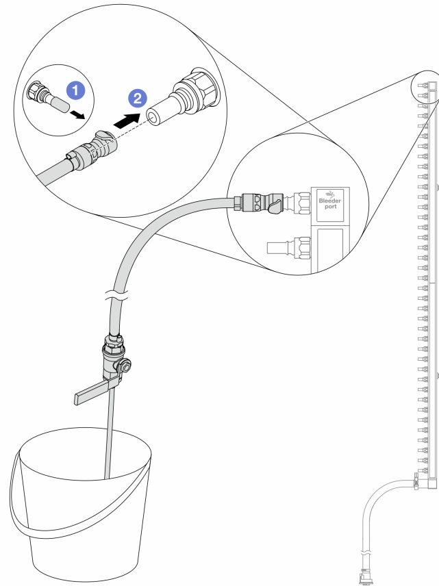
図 165. リターン側へのブリーダー・キットの取り付け
