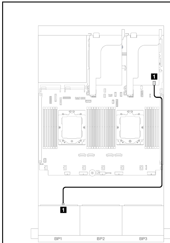
図 380. SAS/SATA ケーブル配線
