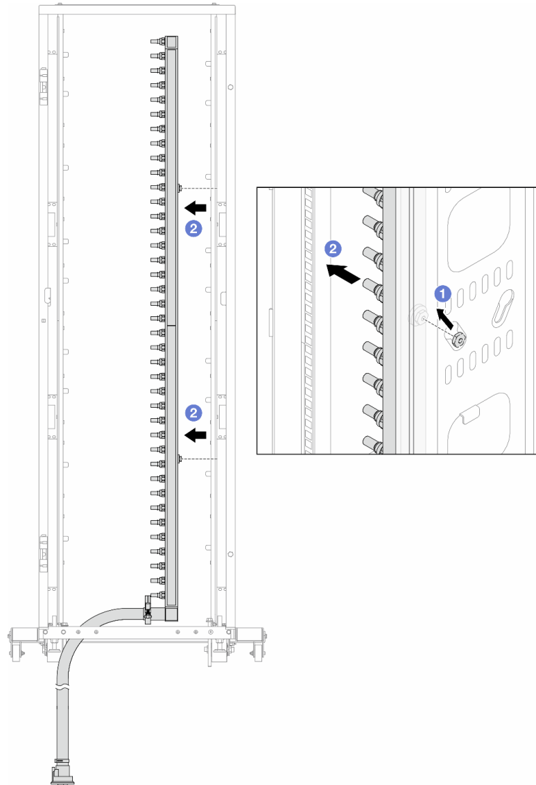
図 162. 多岐管の取り外し
