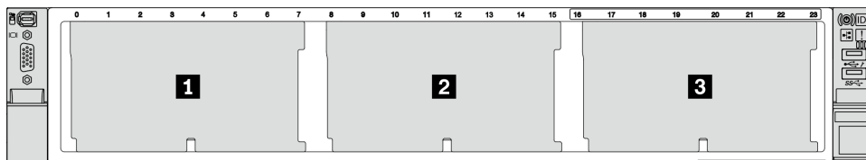
図 72. ドライブ・バックプレーン番号
