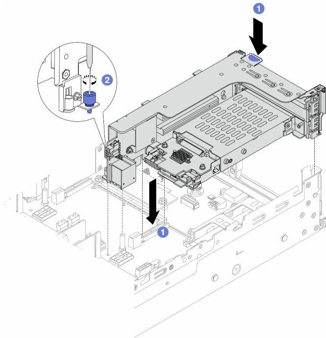
図 241. 2FH+7mm SSD ライザー・ケージの取り付け
