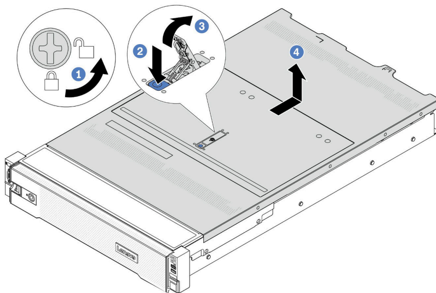
図 309. トップ・カバーの取り外し
