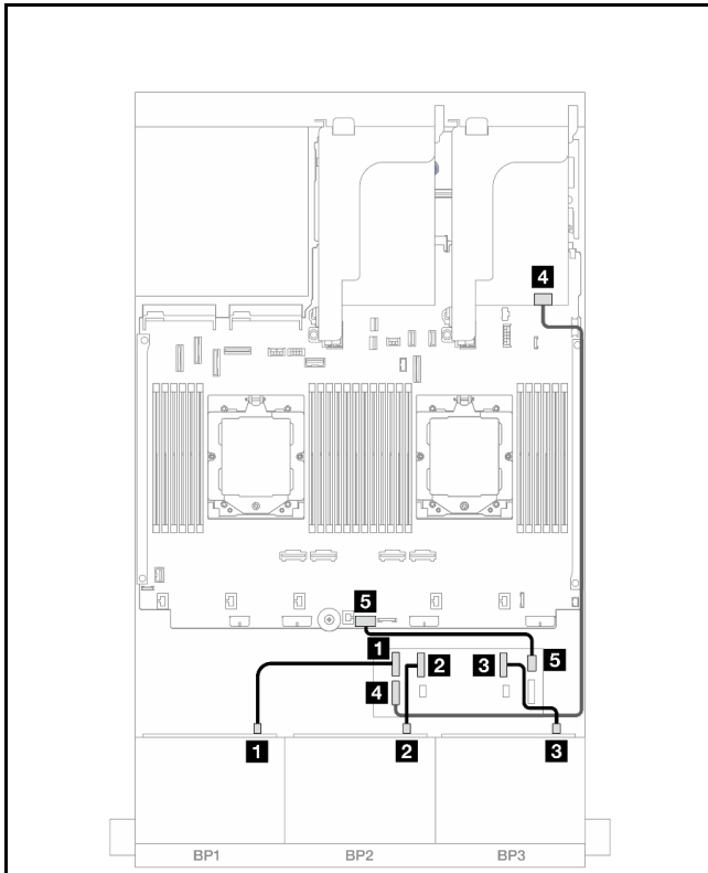
図 464. 前面バックプレーンのケーブル配線
