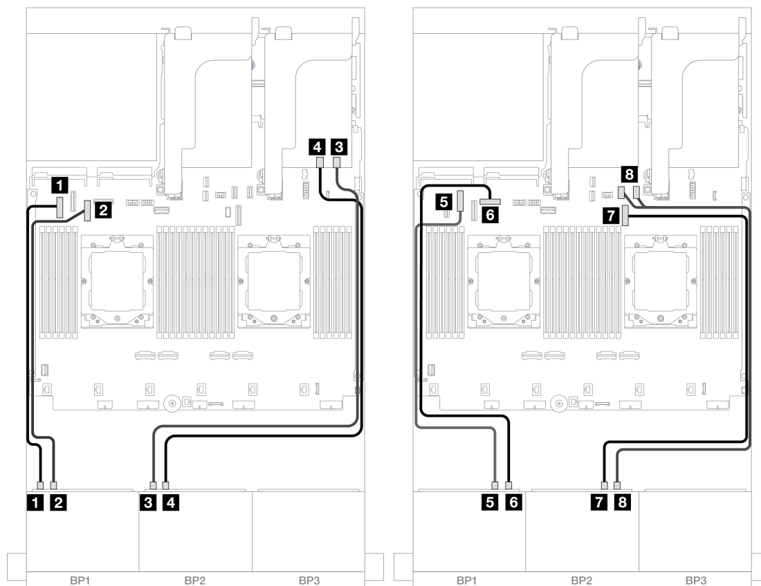
図 436. オンボード・コネクタおよびリタイマー・カードへの NVMe ケーブル配線
