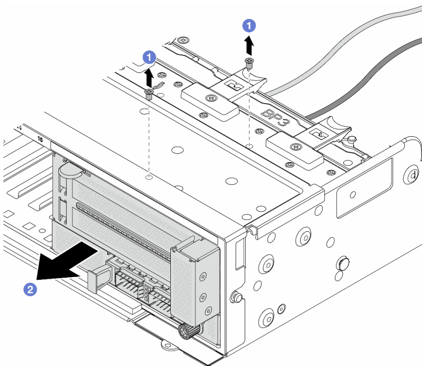
図 62. 前面アダプター・アセンブリーの取り外し
