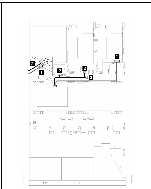
図 396. 中央バックプレーン・ケーブル配線
