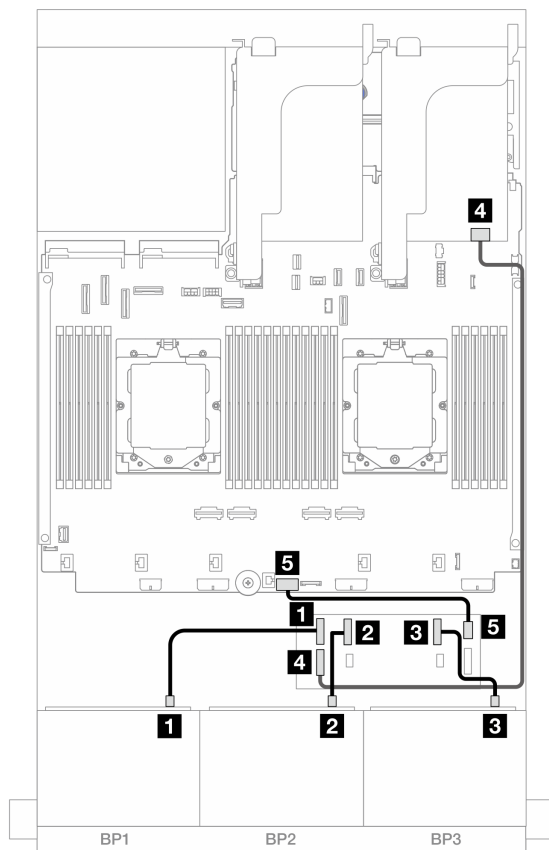
図 479. CFF エクスパンダーおよび 8i/16i アダプターへの SAS/SATA ケーブル配線
