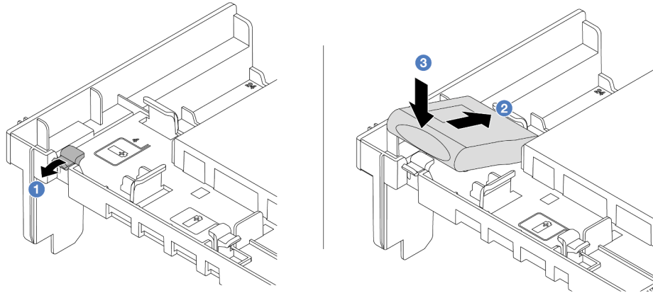
図 219. エアー・バッフルへの RAID フラッシュ電源モジュールの取り付け
