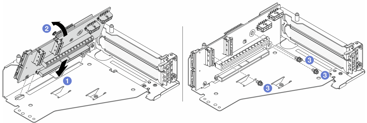
図 66. ライザー・カードの取り付け
