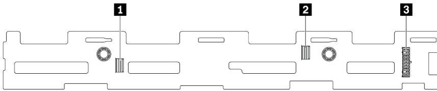
図 314. 8 x 3.5 型 SAS/SATA バックプレーン・コネクタ
