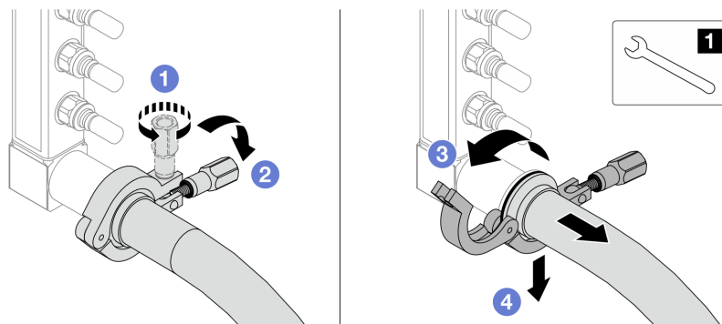
図 167. ホース・キットからの多岐管の分離
