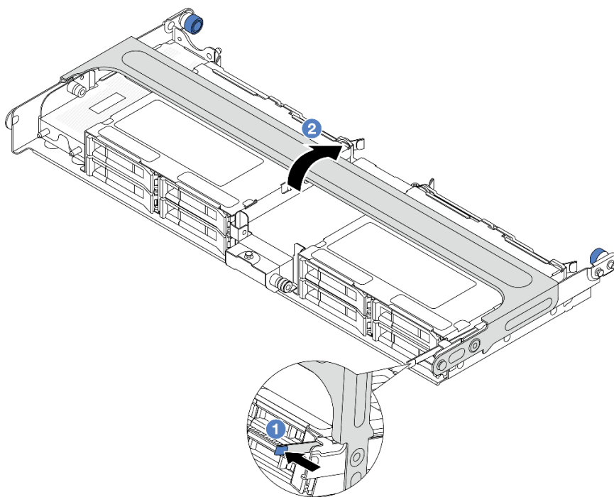
図 224. 中央ドライブ・ケージのハンドルを閉じる
