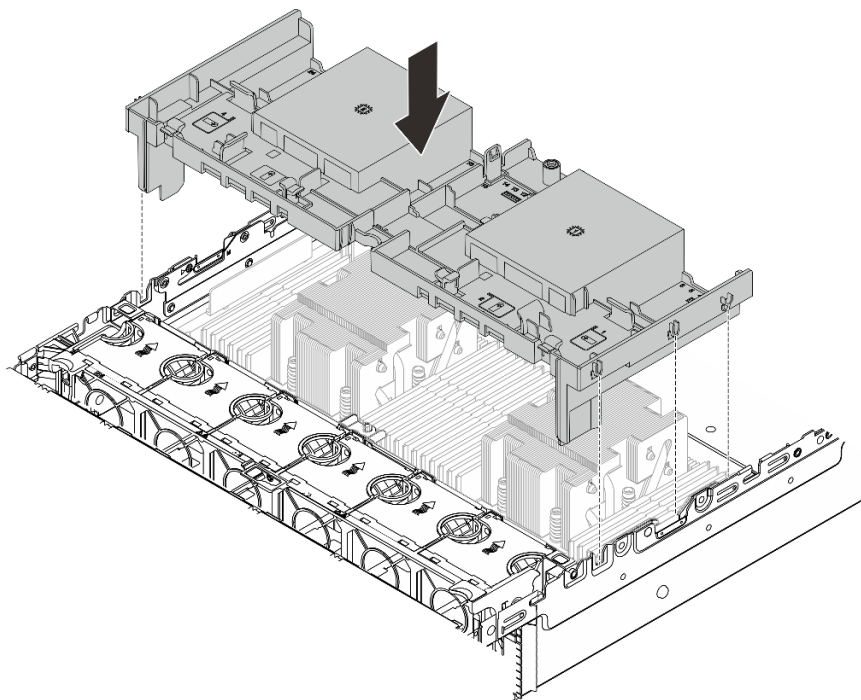
図 33. エアー・バッフルの取り付け
