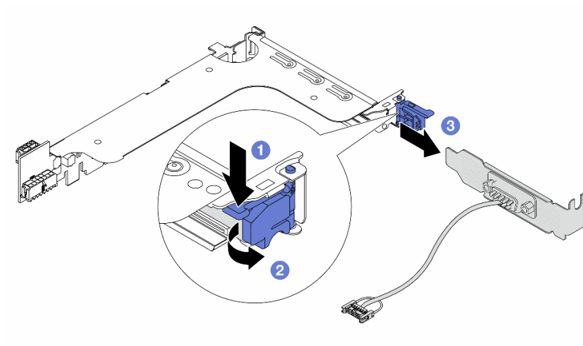
図 304. シリアル・ポート・モジュールの取り外し
