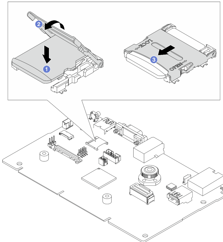
図 182. MicroSD カードの取り付け
