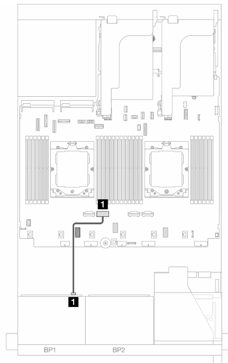
図 381. NVMe ケーブル配線
