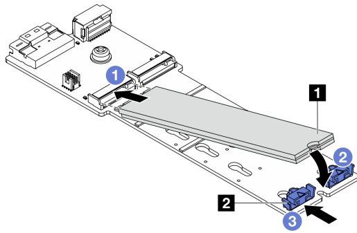
図 117. M.2 ドライブの取り付け
