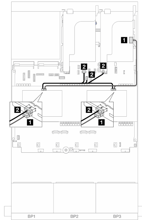
図 474. 中央バックプレーン・ケーブル配線
