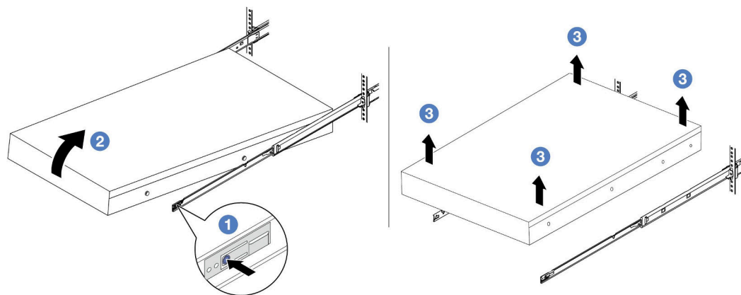
図23. ラックからのサーバーを取り外す。
