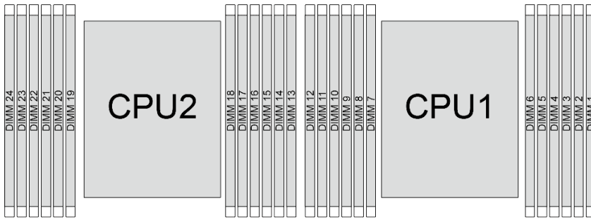
図 19. メモリー・モジュールおよびプロセッサのレイアウト
