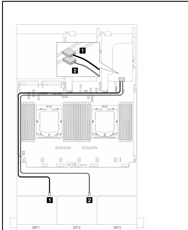
図 524. SAS/SATA ケーブル配線
