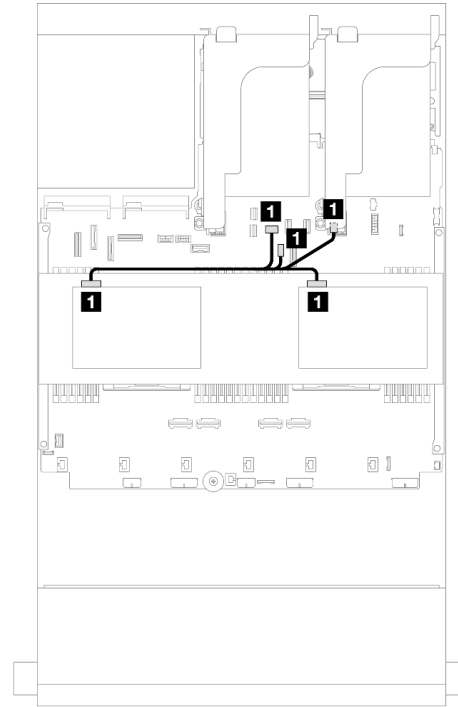
図 562. 中央バックプレーン電源ケーブル配線
