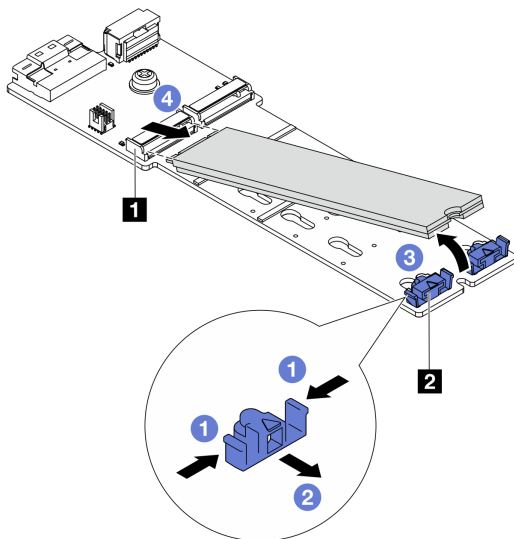
図 114. M.2 ドライブの取り外し
