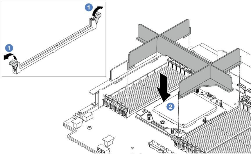
図197. プロセッサ・フィルターの取り付け
