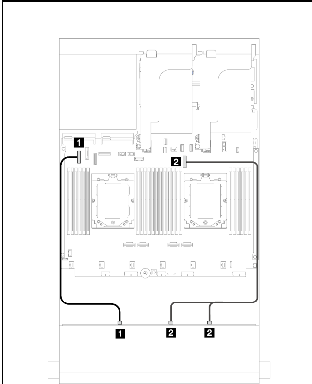
図 544. 2つのプロセッサが取り付け済みである場合のオンボード SATA コネクタへのケーブル配線
