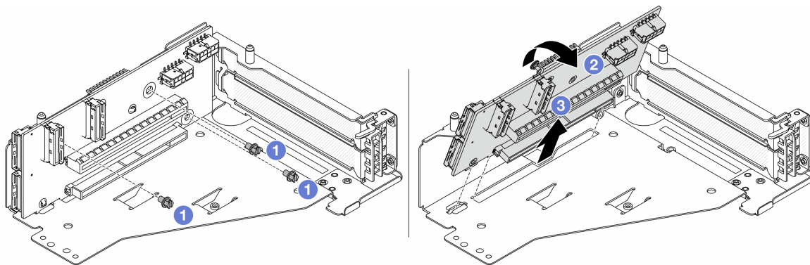
図 65. ライザー 5 ケージからのライザー・カードの取り外し
