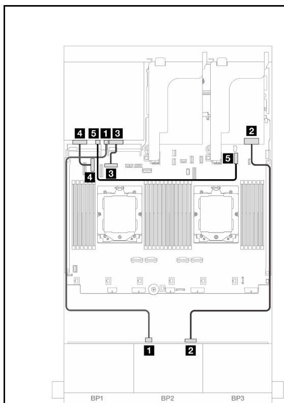
図534. 2つのプロセッサが取り付けられた場合のケーブル配線
