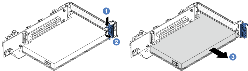
図269. ライザー 3 アセンブリーからの PCIe アダプターの取り外し
