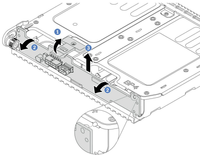
図 252. 2 x 3.5 型背面ドライブ・バックプレーンの取り外し
