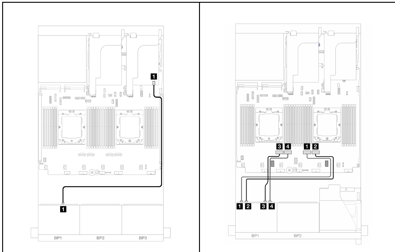
図 370. SAS/SATA ケーブル配線
