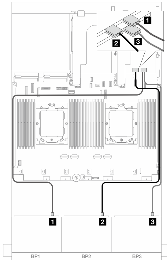
図 439. 8i/16i アダプターへの SAS/SATA ケーブル配線
