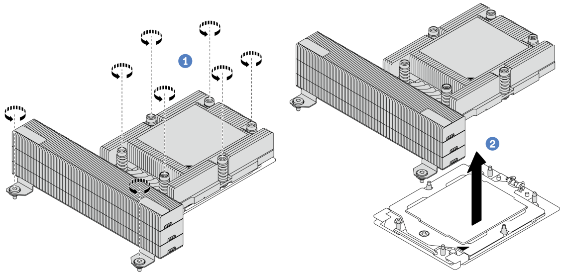
図 195. パフォーマンス・ヒートシンクの取り外し
