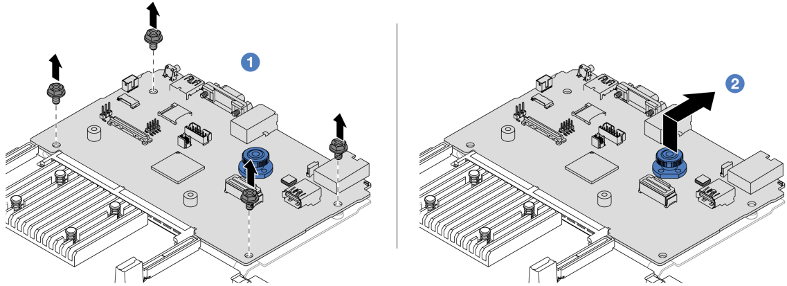
図 293. システム I/O ボードのプロセッサ・ボードからの取り外し
