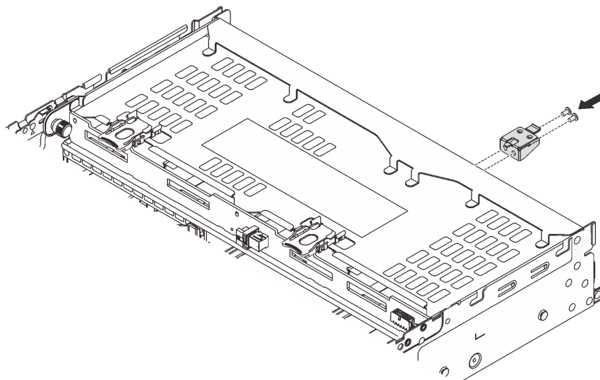
図 259. トップ・カバー・サポート・ブラケットの取り付け
