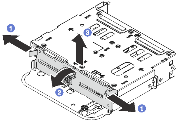
図244. 4 x 2.5 型背面ドライブ・バックプレーンの取り外し
