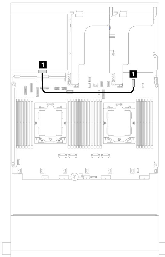
図 557. 背面バックプレーン電源ケーブルの配線
