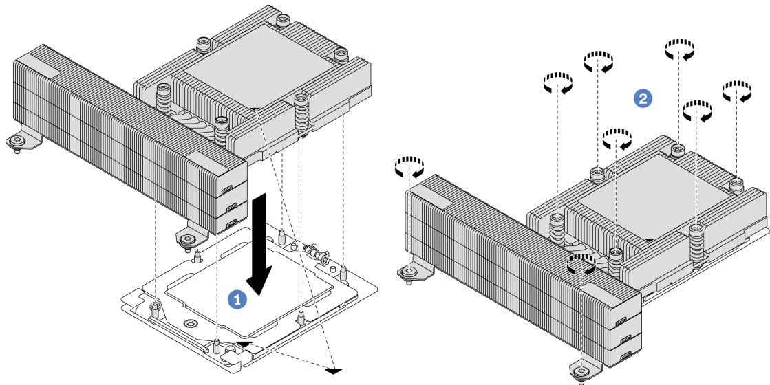
図 202. パフォーマンス・ヒートシンクの取り付け
