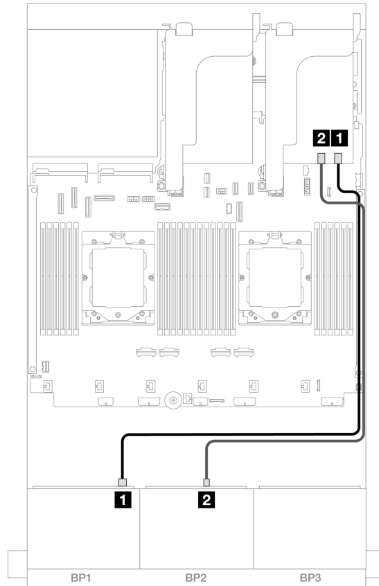
図 409. 16i アダプターへの SAS/SATA ケーブル配線
