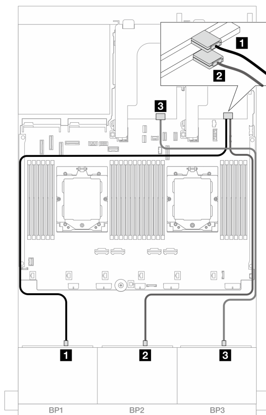
図 489. 8i Trimode アダプターへの SAS/SATA ケーブル配線
