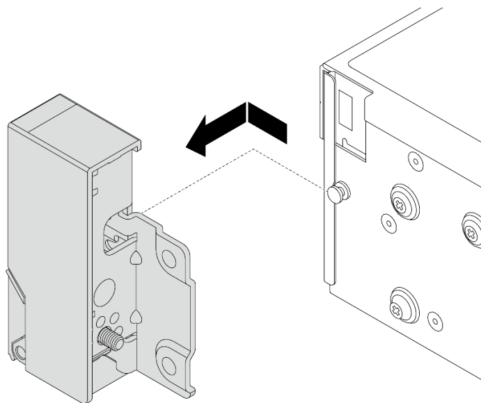
図 206. ラック・ラッチの取り外し
