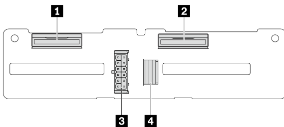
図 323. 4 x 2.5 型 AnyBay バックプレーン・コネクタ
