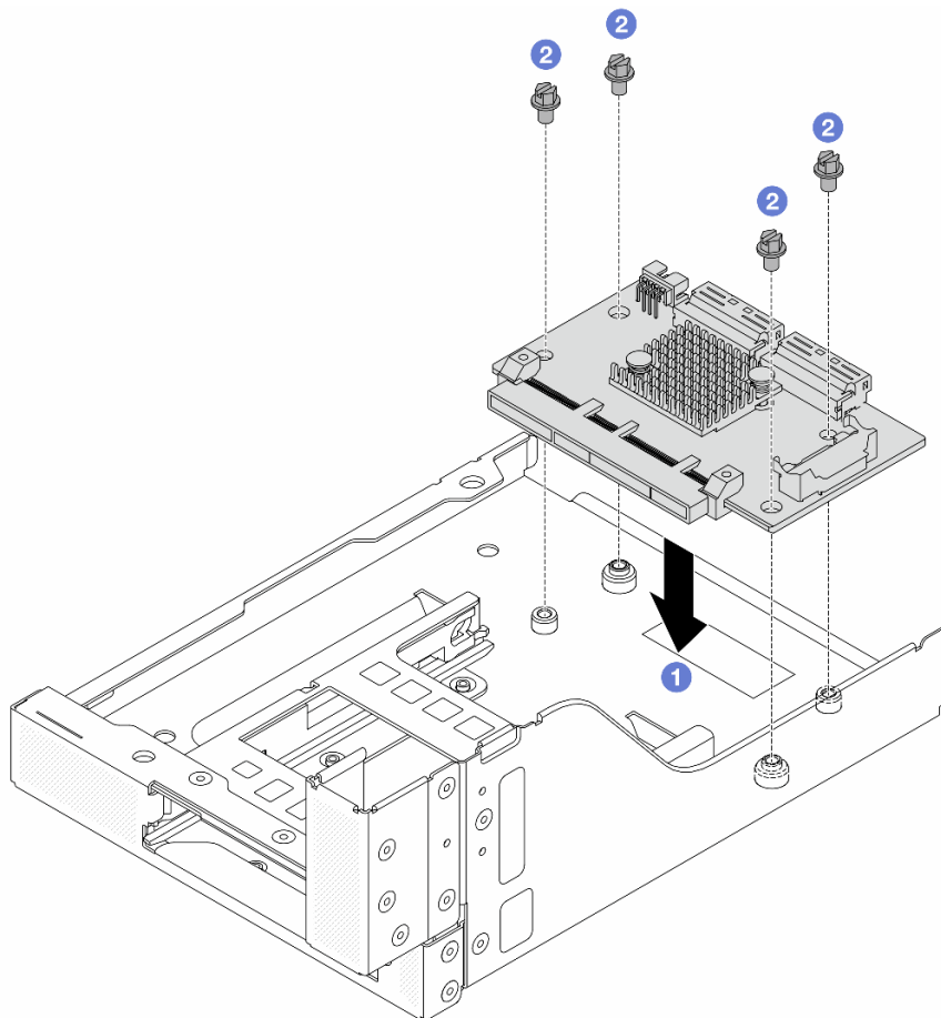
図 56. 前面 OCP 変換コネクタ・カードの取り付け
