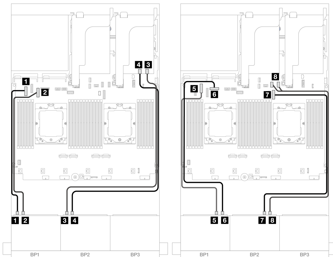
図 405. オンボード・コネクターおよびリタイマー・カードへの NVMe ケーブル配線
