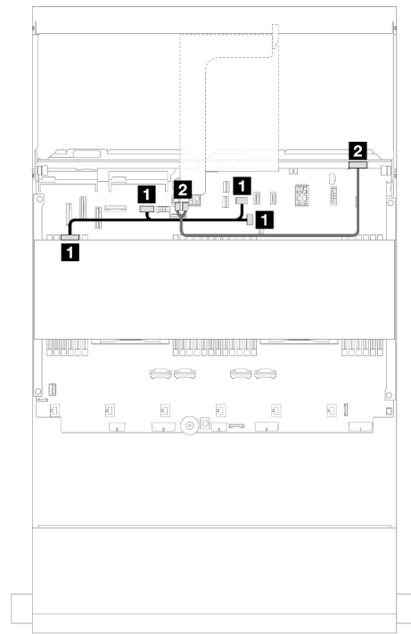
図 586. 中央/背面バックプレーン電源ケーブル配線
