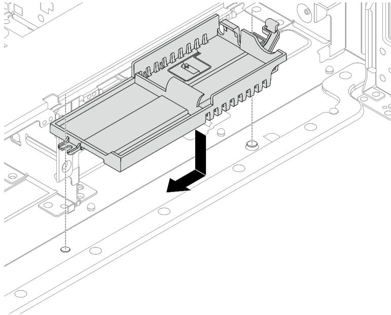
図 216. スーパーキャップ・ホルダーの取り付け
