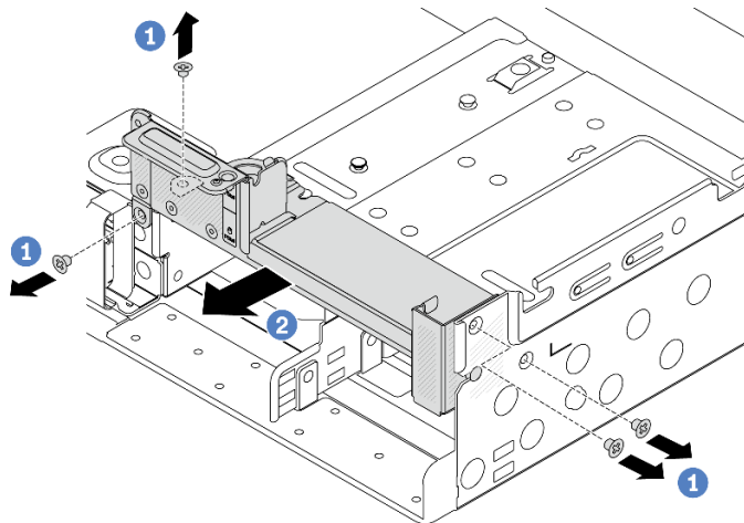
図 228. C1 背面壁ブラケットの取り外し(右)
