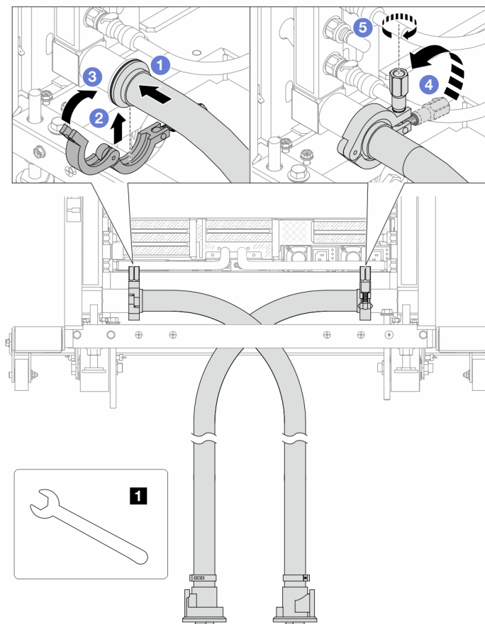
図 170. ホース・キットの取り付け
