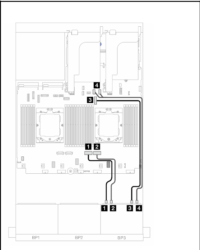
図 527. NVMe ケーブル配線
