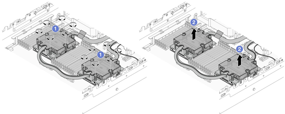
図104. DWCM の取り外し
