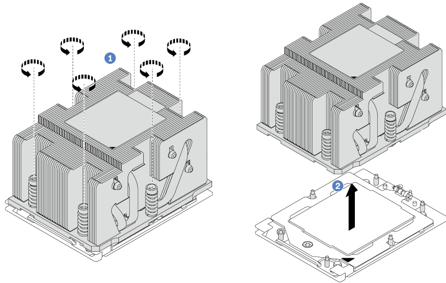
図 194. 標準ヒートシンクの取り外し
