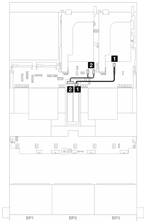
図 335. SATA/NVMe のケーブル配線
