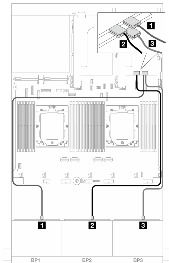
図 490. 8i/16i Trimode アダプターへの SAS/SATA ケーブル配線
