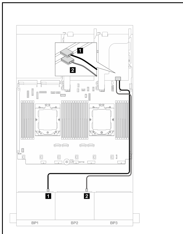
図 522. SAS/SATA ケーブル配線
