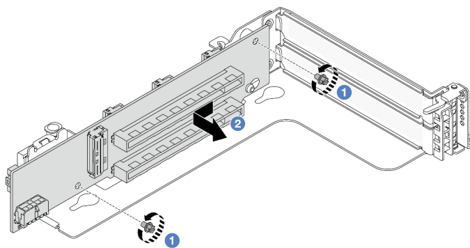
図 272. ライザー 3 ケージからのライザー・カードの取り外し
