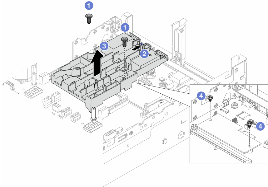
図 105. ホース・ホルダーの取り外し
