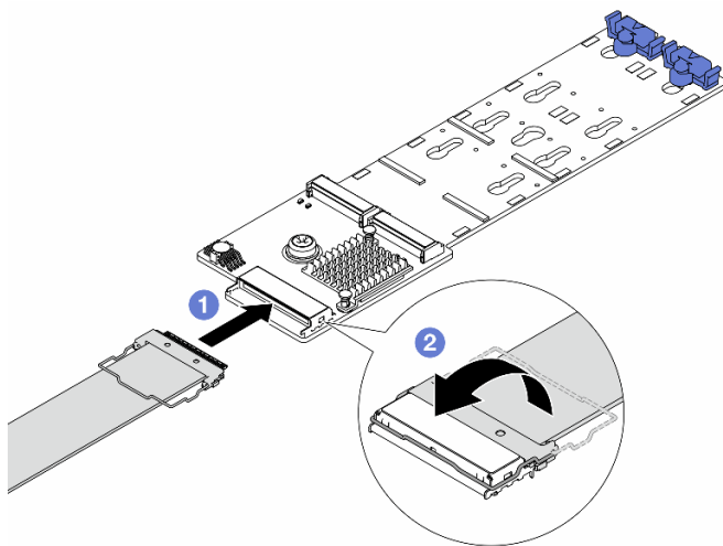
図 129. M.2 ケーブルの M.2 RAID SATA/NVMe 2 ベイ・バックプレーン への接続
