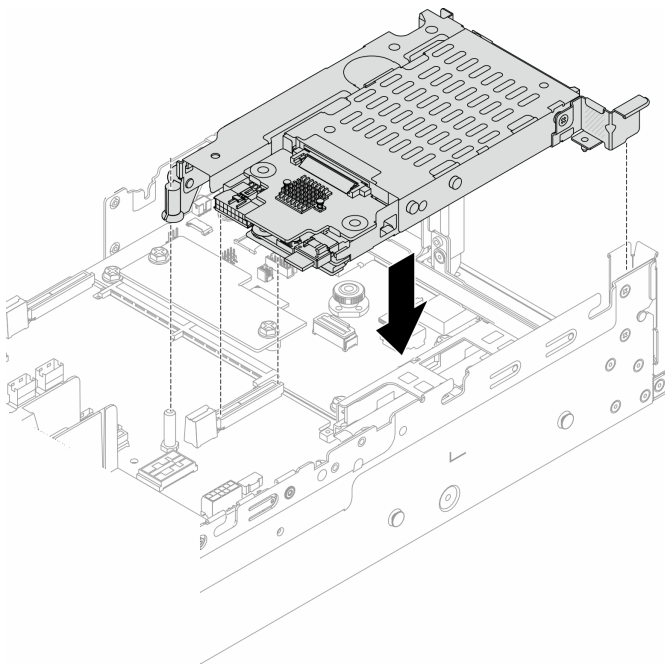
図 242. 7mm SSD ライザー・ケージの取り付け
