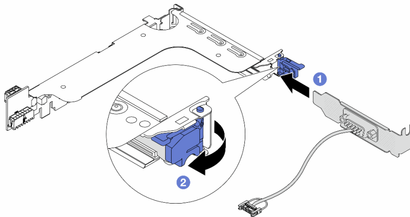
図 307. シリアル・ポート・モジュールの取り付け
