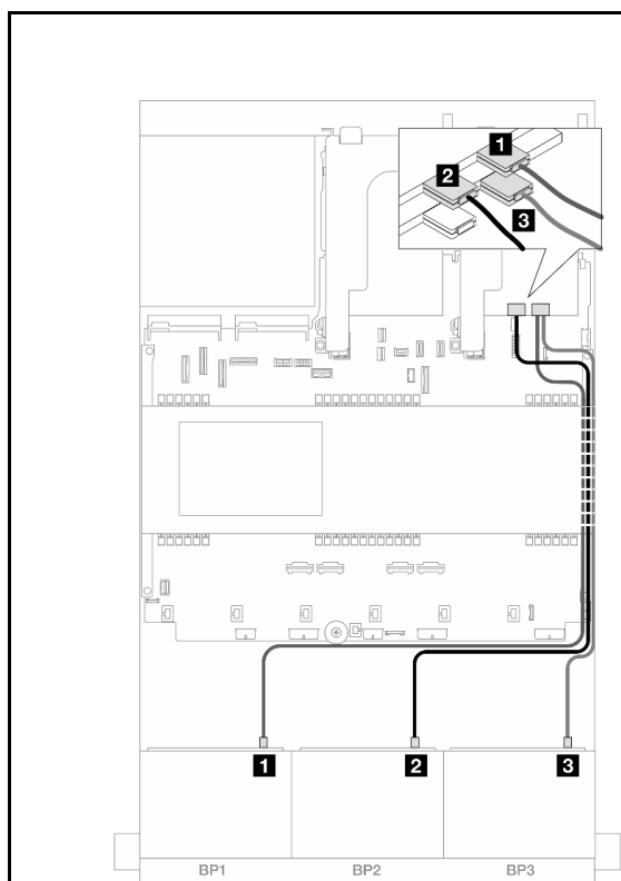
図 459. 前面バックプレーンのケーブル配線
