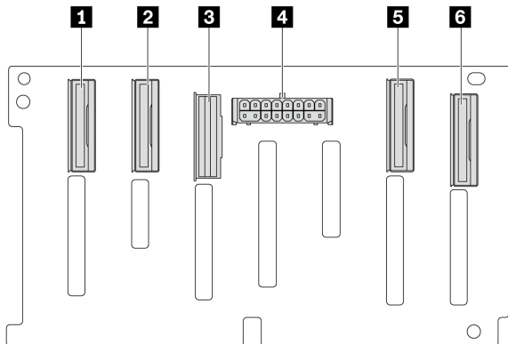
図 312. 8 個の 2.5 型 AnyBay バックプレーン・コネクタ
