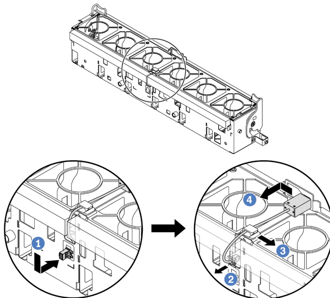
図99. 侵入検出スイッチの取り外し
