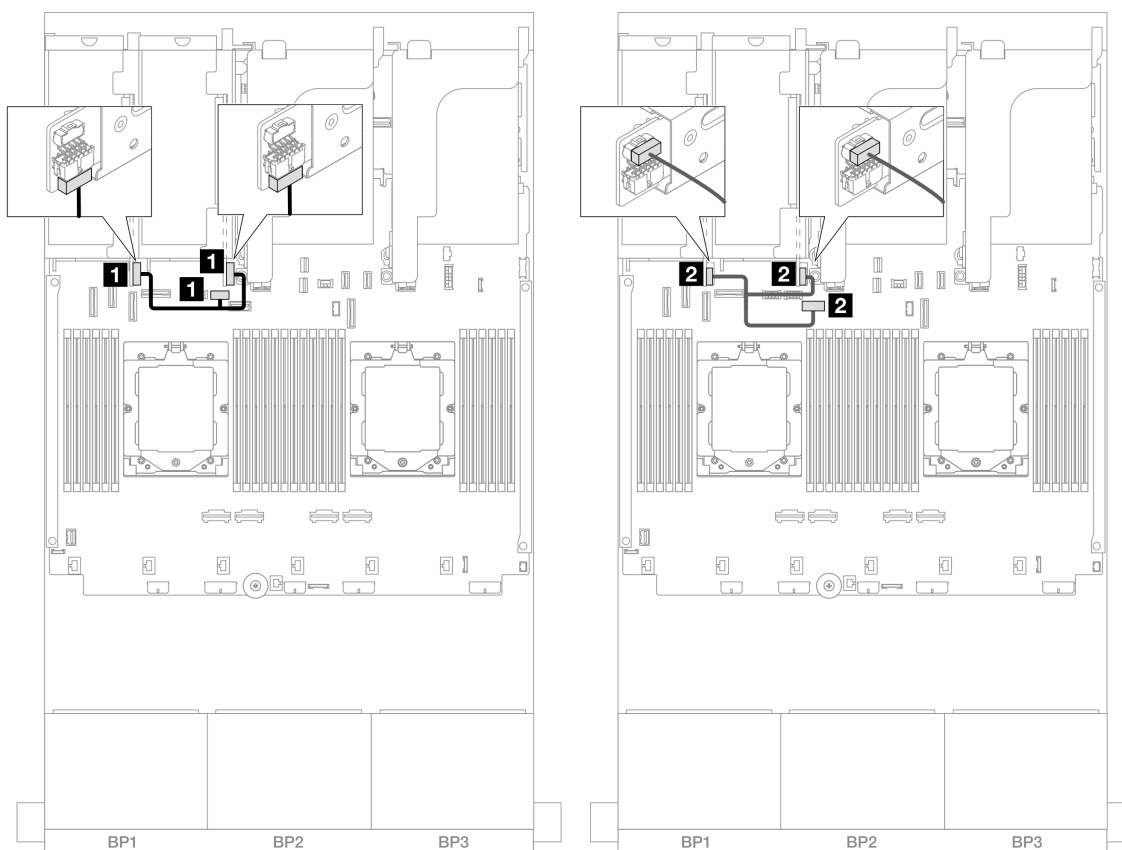
図 353. ライザー・カード 3/4 電源および側波帯ケーブル配線
