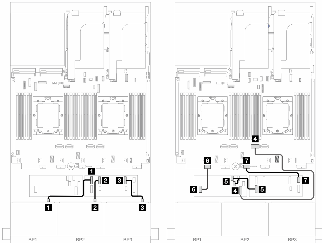
図 482. CFF エクスパンダーおよび CFF 16i アダプターへの SAS/SATA ケーブル配線
