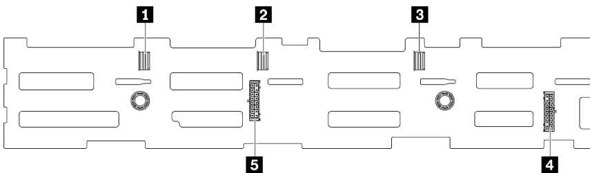
図 315. 12 個の 3.5 型 SAS/SATA バックプレーン・コネクタ
