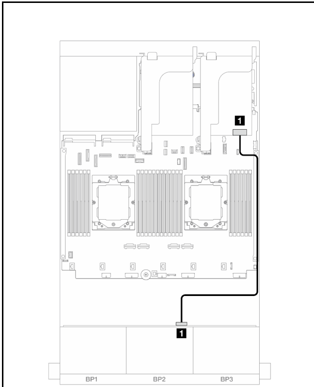
図 536. 前面バックプレーンのケーブル配線
