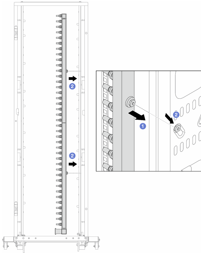
図 168. 多岐管の取り付け
