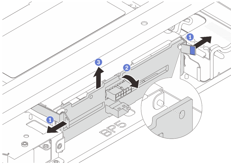
図184. 中央 2.5 型ドライブ・バックプレーンの取り外し
