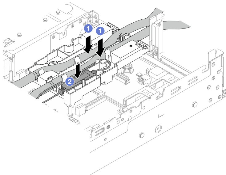
図110. ホースおよびモジュールの取り付け
