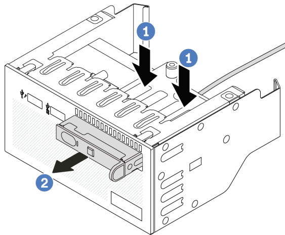
図 80. 内蔵診断パネルの取り外し
