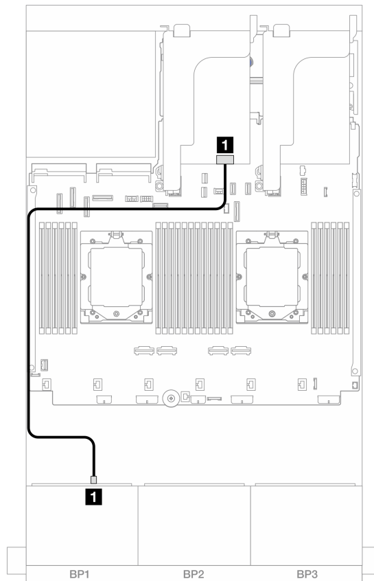
図 497. 8i アダプターへの SAS/SATA ケーブル配線
