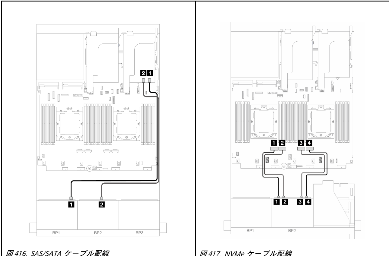
図 416. SAS/SATA ケーブル配線
