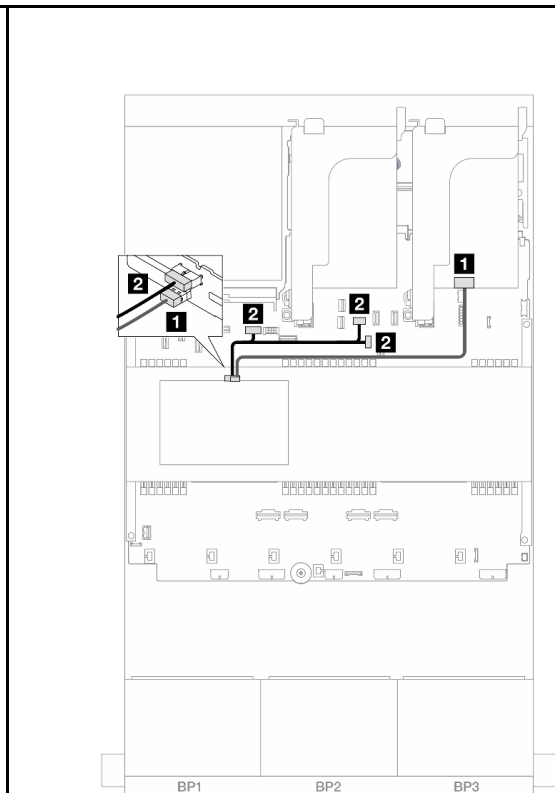
図 472. 中央バックプレーン・ケーブル配線
