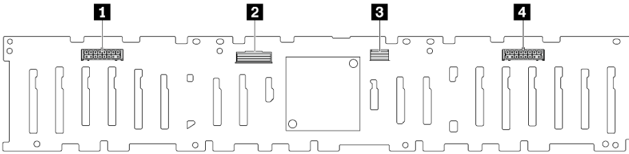
図 313. 24 x 2.5 型 SAS/SATA エクspander・バックプレーン上のコネクタ
