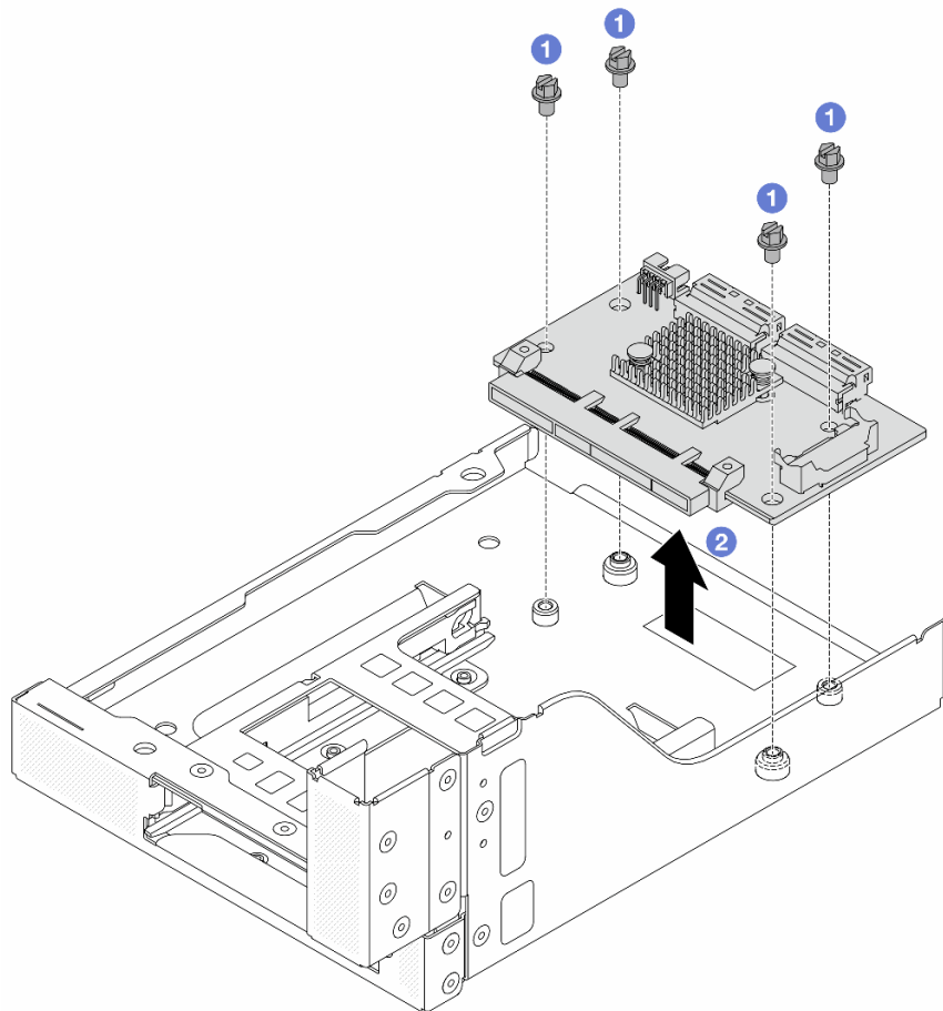
図 55. 前面 OCP 変換コネクタ・カードの取り外し
