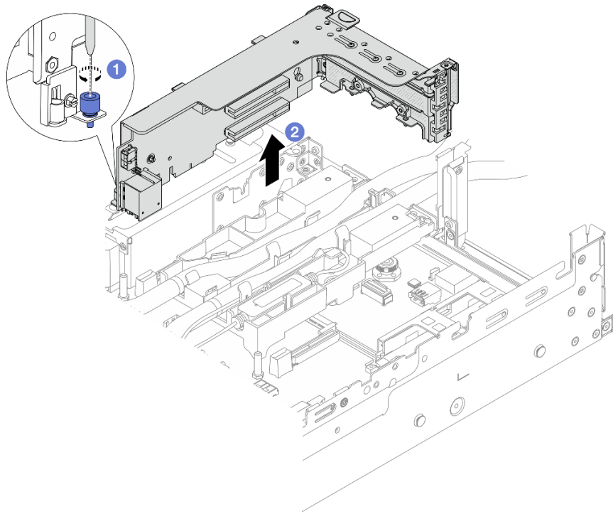
図 102. 3FH ライザー・ケージの取り外し
