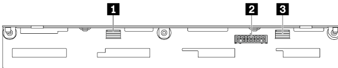
図 322. 8x2.5 型 SAS/SATA バックプレーン・コネクタ
