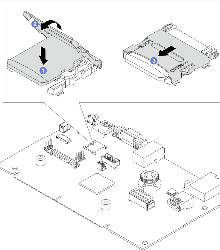
図 295. MicroSD カードの取り付け
