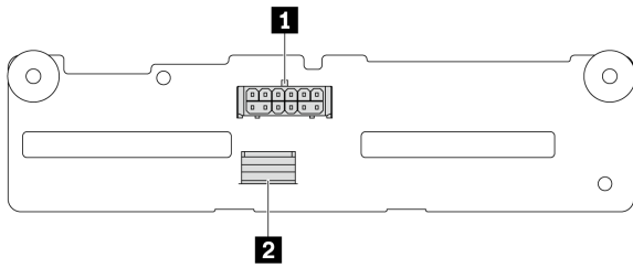
図 318. 4 個の 2.5 型 SAS/SATA バックプレーン・コネクタ
