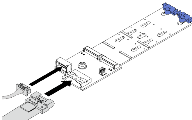
図 127. M.2 ケーブルの M.2 x4 非 RAID SATA/NVMe 2 ベイ・バックプレーン への接続
