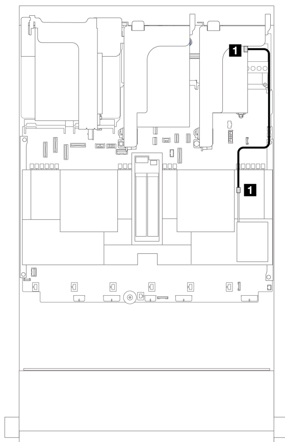
図 345. RAID フラッシュ電源モジュールのケーブル配線
