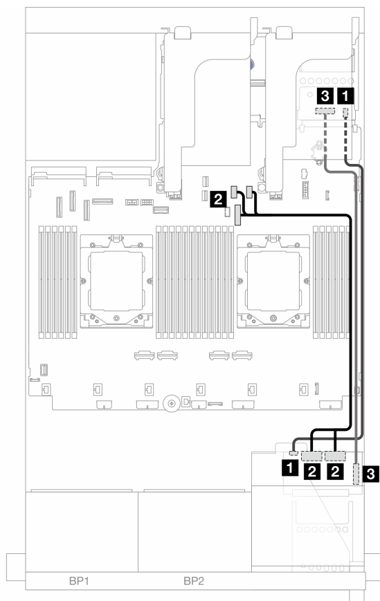
図 340. OCP 変換コネクタ・カードのケーブル配線
