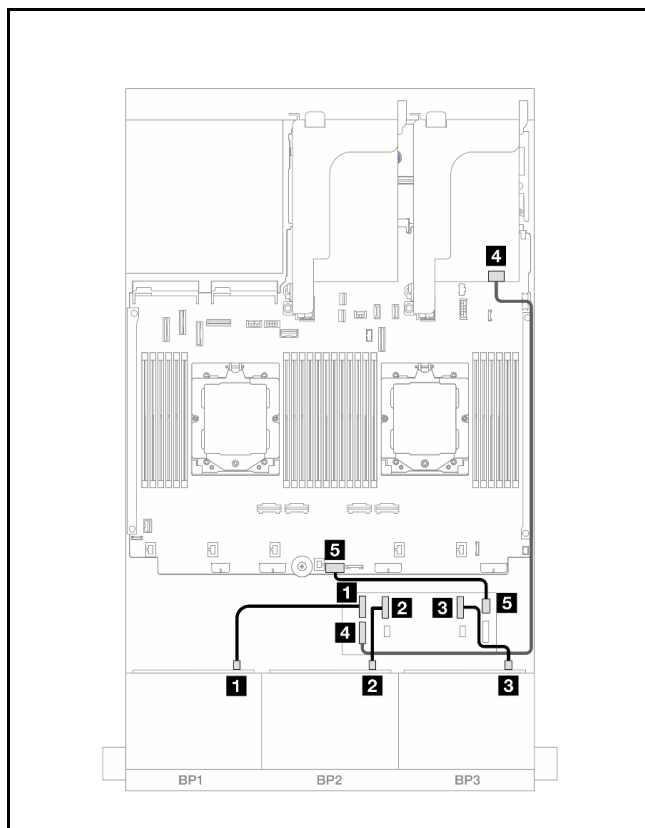
図 442. 前面バックプレーンのケーブル配線
