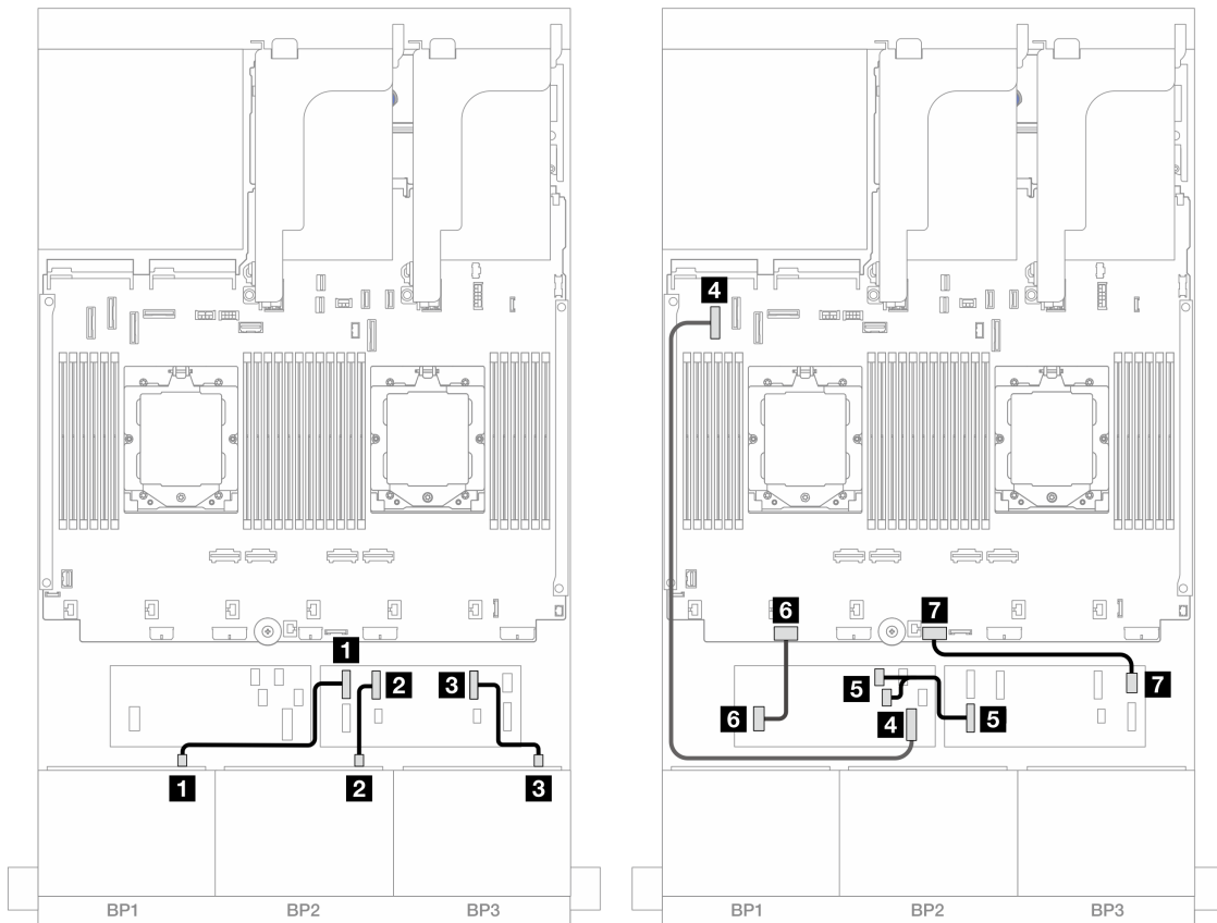
図 444. CFF エクスパンダーおよび CFF 16i アダプターへの SAS/SATA ケーブル配線
