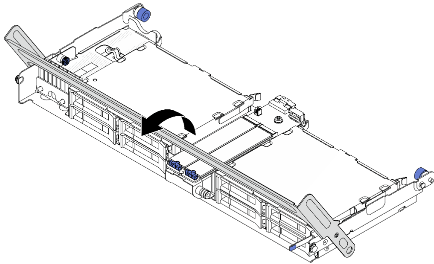
図 122. 中央ドライブ・ケージのハンドルを開く
