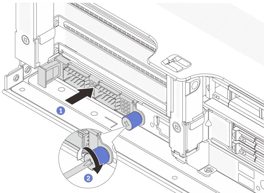
図 261. 背面 OCP モジュールの取り付け
