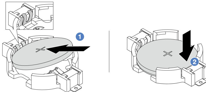
図 37. CMOS バッテリーの取り付け
