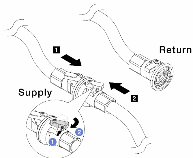
図 175. ファシリティー供給から多岐管の供給へ
