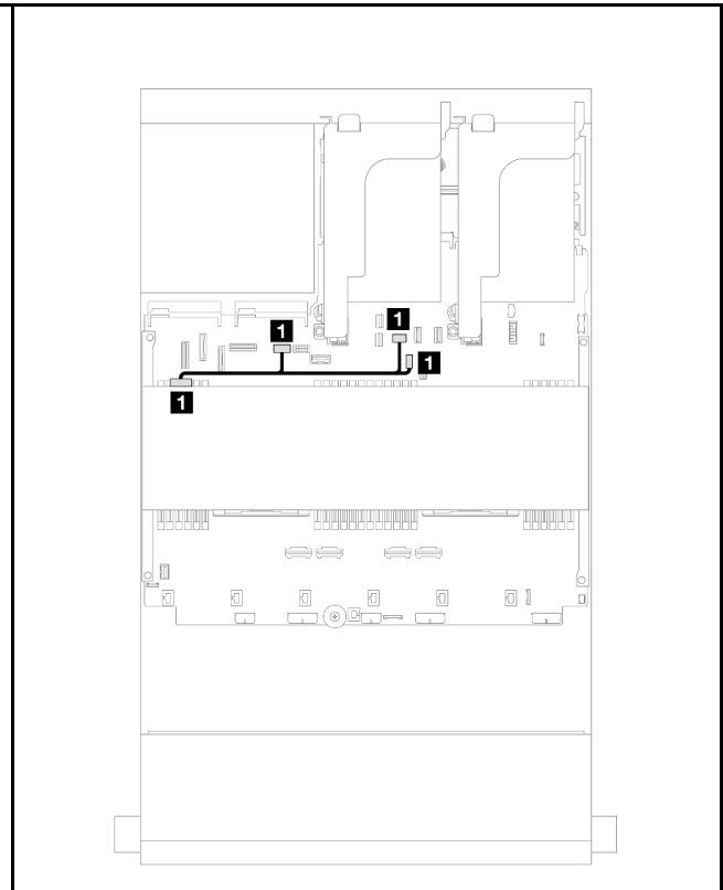
図 559. 中央バックプレーン電源ケーブル配線
