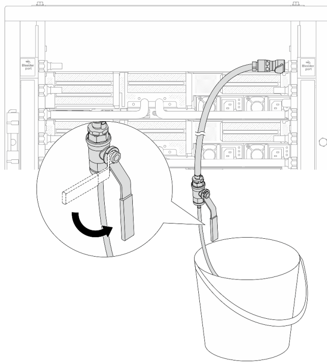
図 176. リターン側のブリーダー・バルブを開く
