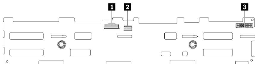
図 316. 12 x 3.5 型 SAS/SATA エクスパンダー・バックプレーン上のコネクタ
