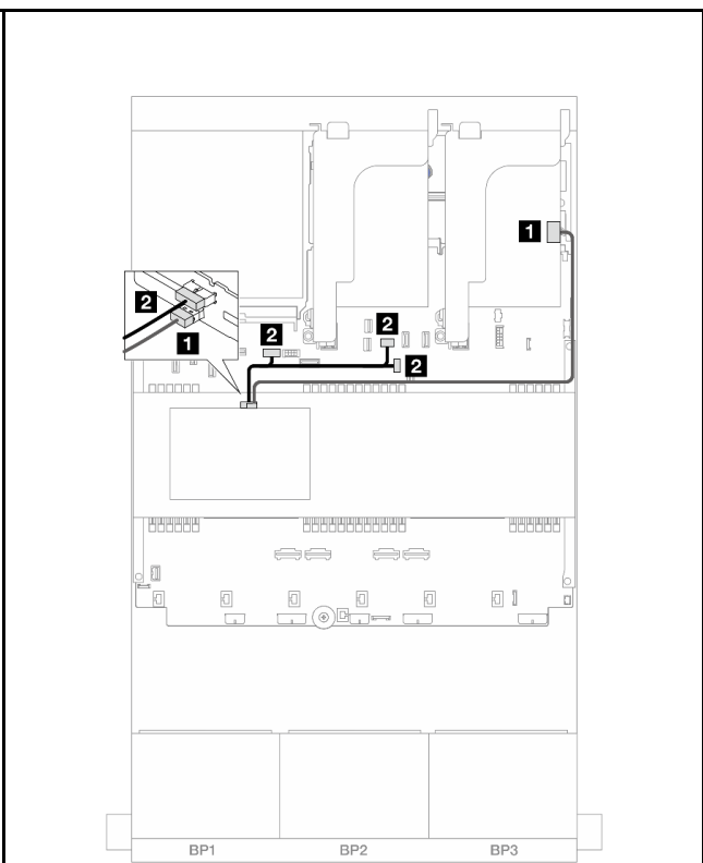
図 470. 中央バックプレーン・ケーブル配線
