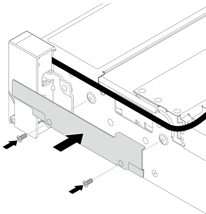
図 209. ケーブル保持具の取り付け
