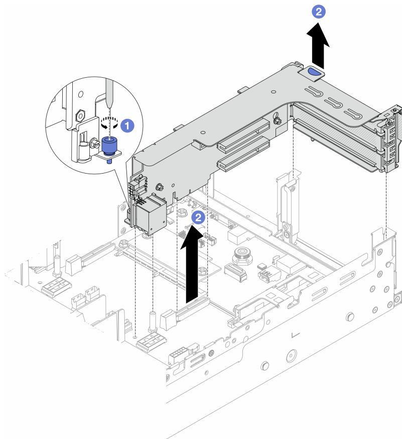
図 264. ライザー・アセンブリー 1 の取り外し
