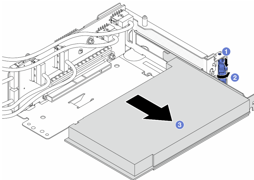
図 40. PCIe ライザー 5 ケージからの PCIe アダプターの取り外し
