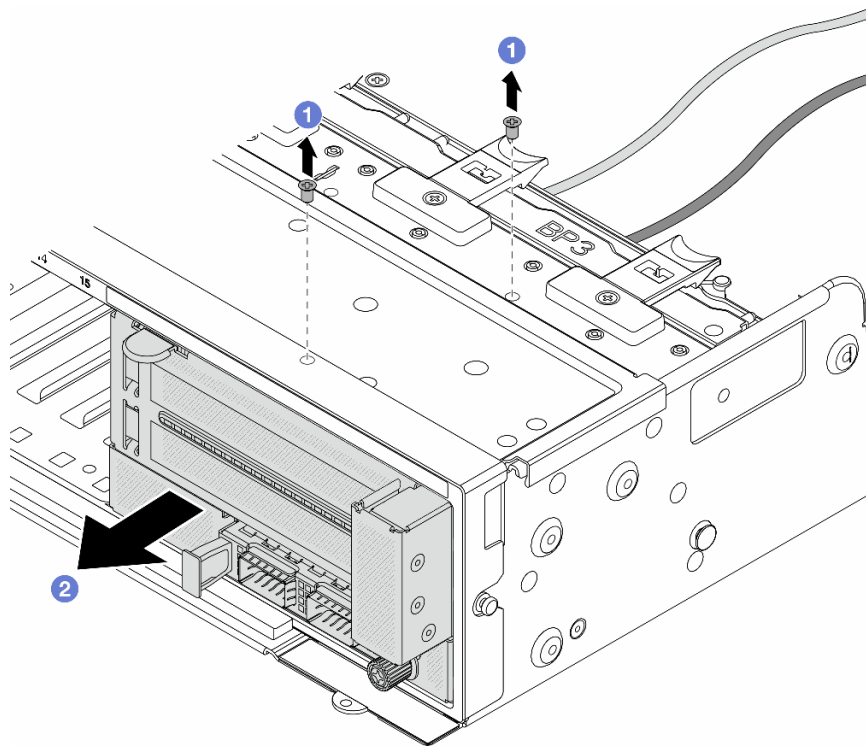
図 38. 前面アダプター・アセンブリーの取り外し
