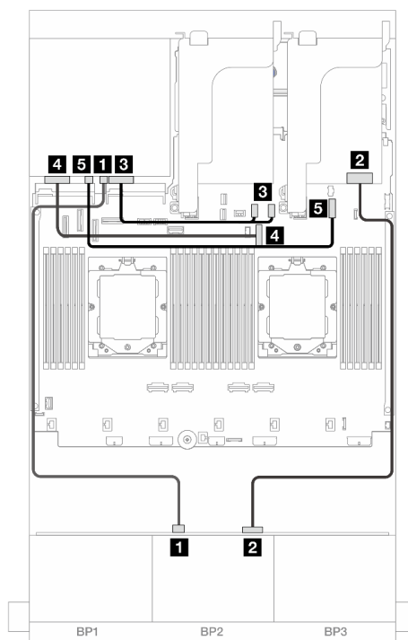
図535. 1つのプロセッサが取り付けられた場合のケーブル配線
