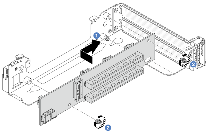
図275. ライザー 3 ケージへのライザー・カードの取り付け
