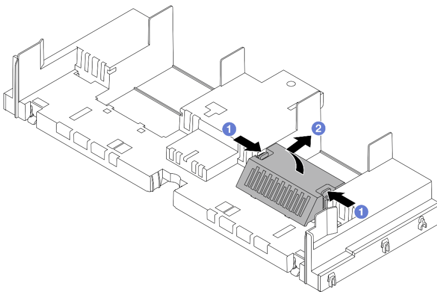
図 31. エアー・バッフル・フィラーの取り外し
