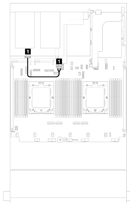
図 581. 背面バックプレーン電源ケーブルの配線
