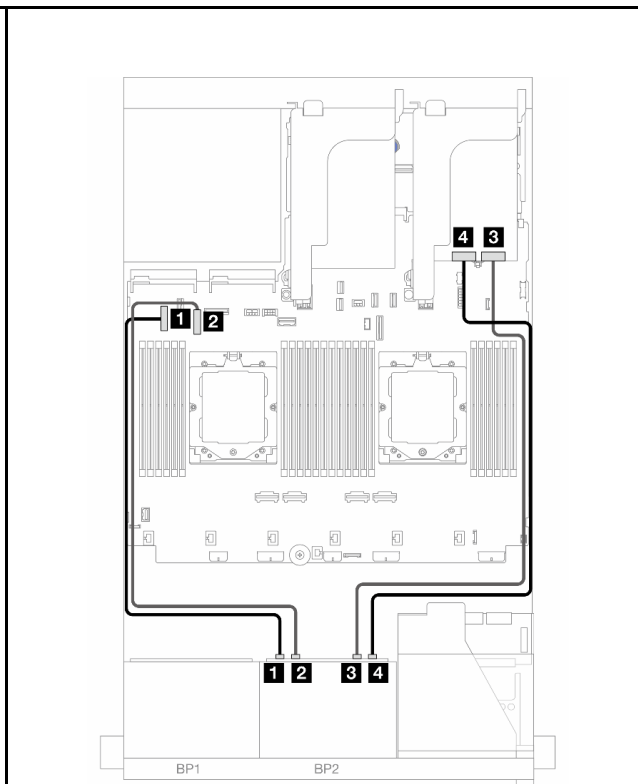
図 419. NVMe ケーブル配線
