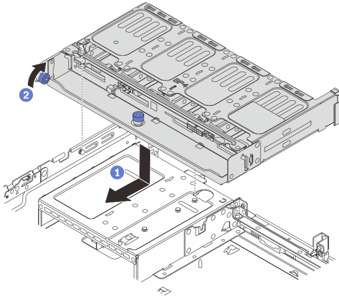
図 250. 8 x 2.5 型背面ドライブ・ケージの取り付け
