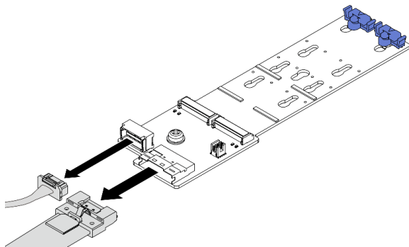
図 118. M.2 x4 非 RAID SATA/NVMe 2 ベイ・バックプレーンからのケーブルの取り外し
