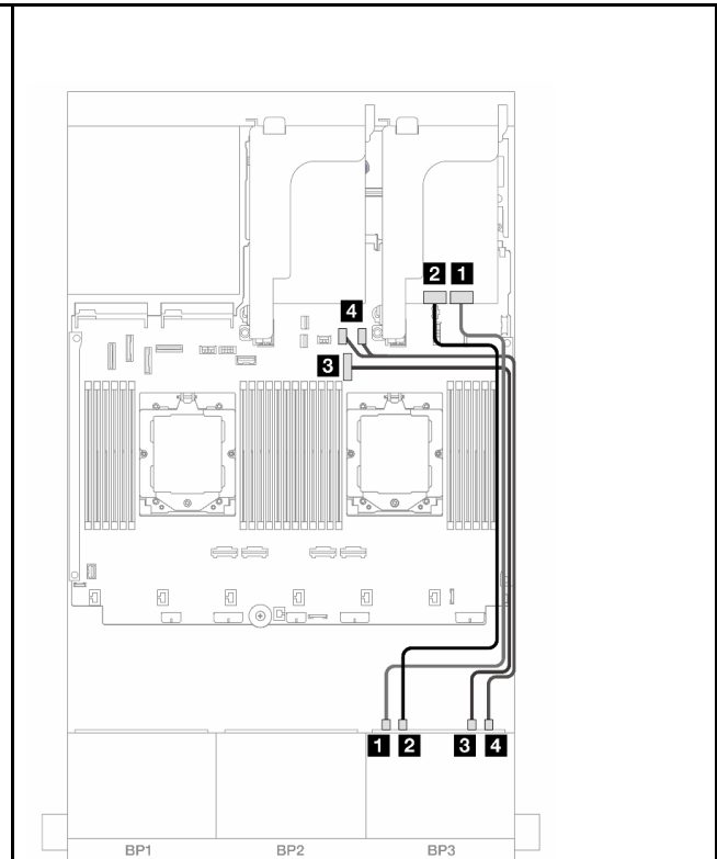
図 525. NVMe ケーブル配線
