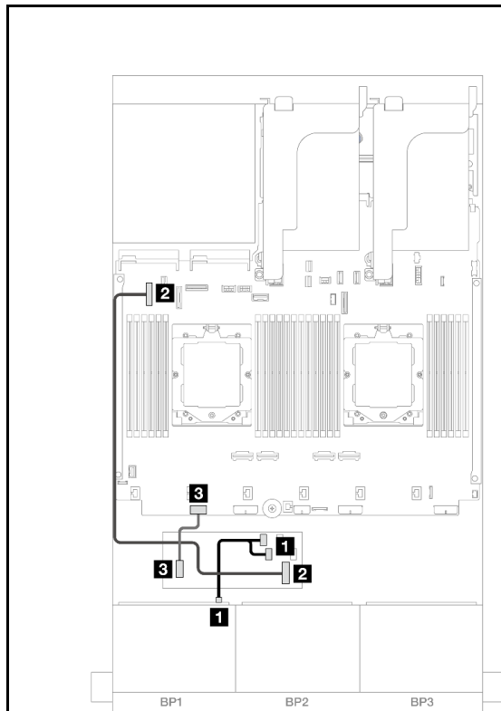
図363. 2つのプロセッサが取り付けられた場合のケーブル配線
