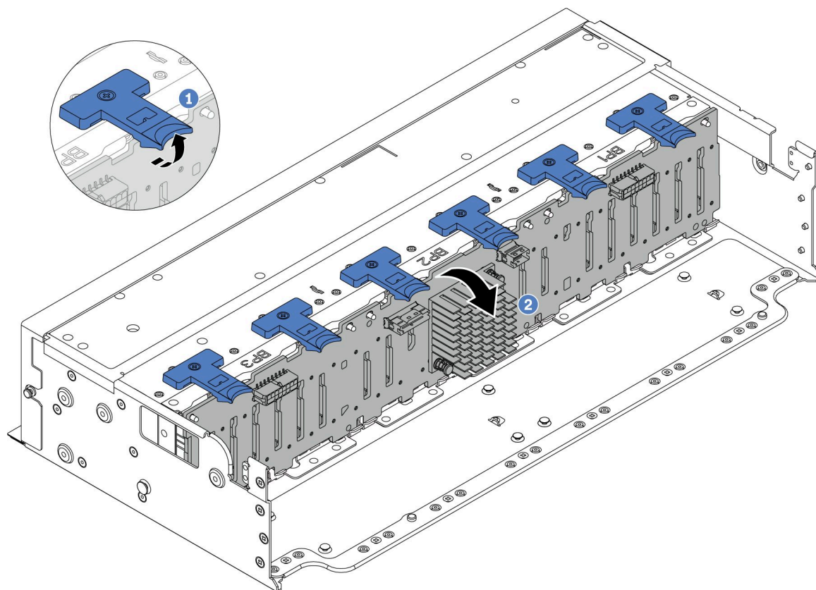
図 71. 24 ベイ・ドライブ・バックプレーンの取り外し
