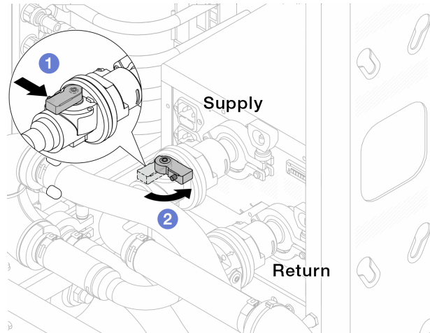
図 138. ボール・バルブを閉じる
