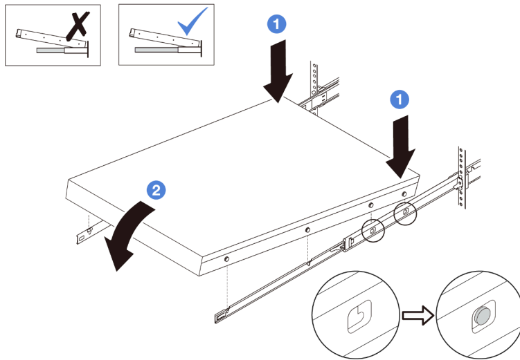
図 26. サーバーをラックに取り付ける
