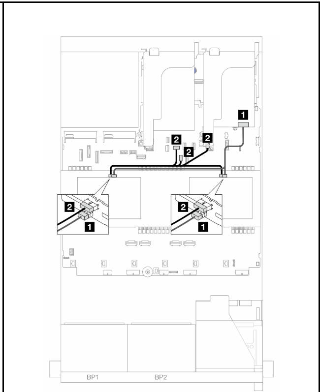
図 398. 中央バックプレーン・ケーブル配線
