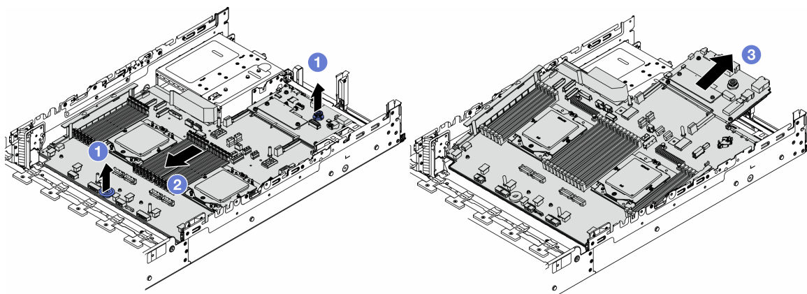
図 292. システム・ボード・アセンブリーの取り外し
