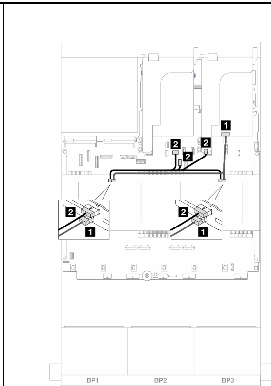
図 476. 中央バックプレーン・ケーブル配線
