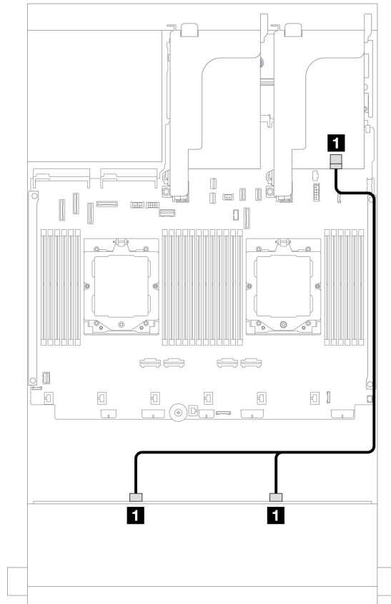
図 543. 8i RAID/HBA アダプターへのケーブル配線
