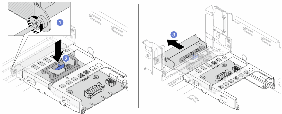
図 60. 背面 OCP 変換コネクタ・カードの取り外し
