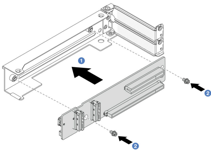
図276. 4LP ライザー 3/4 ケージへのライザー・カードの取り付け
