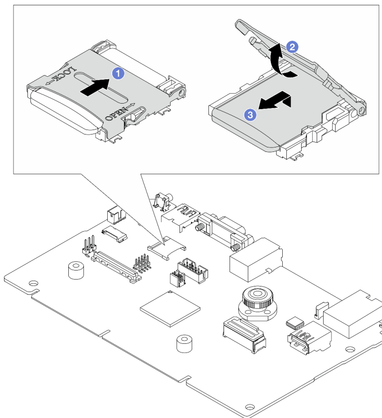
図 294. MicroSD カードの取り外し
