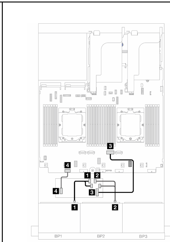
図 392. 1つのプロセッサが取り付けられた場合のケーブル配線
