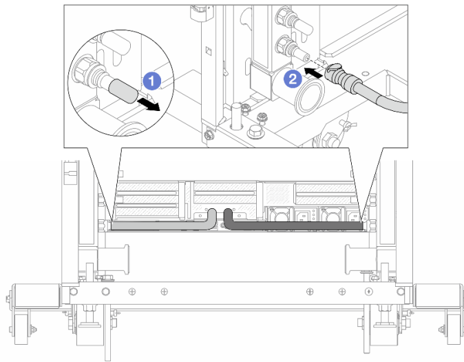
図 169. クイック・コネクト・プラグの取り付け
