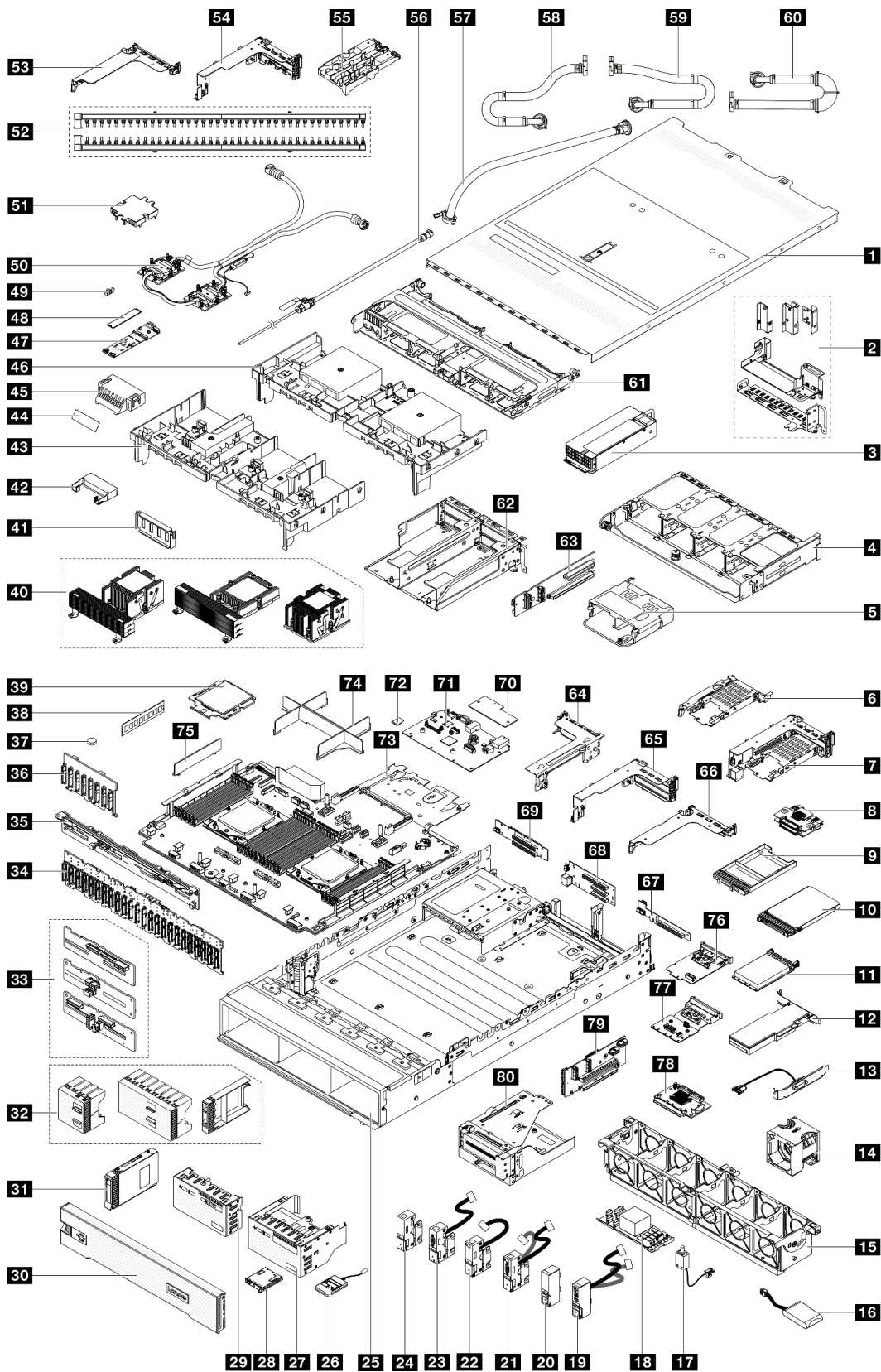
図 14. サーバー・コンポーネント (2.5 型ドライブ・ベイのシャーシ)
