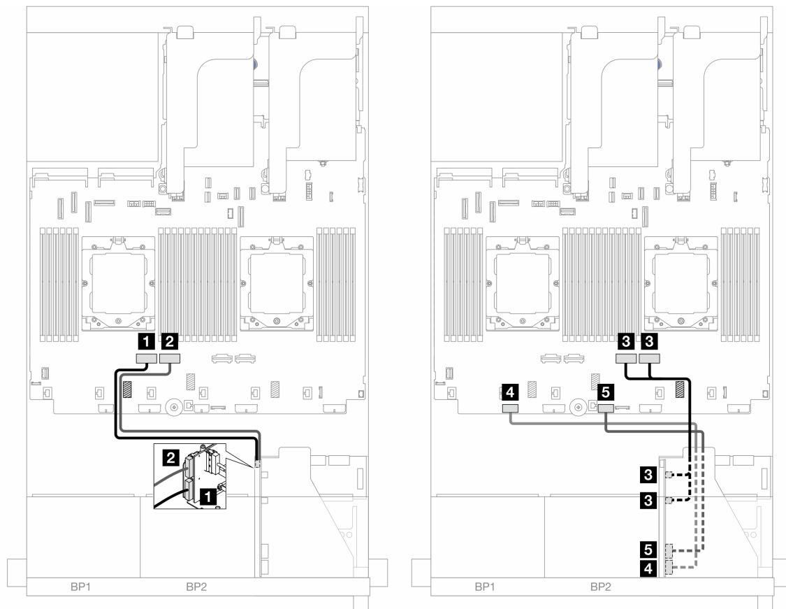
図 356. ライザー 3/4 のある構成のケーブル配線
