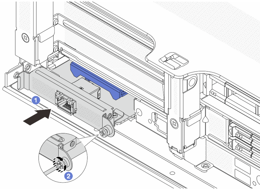
図 131. 管理 NIC アダプターの取り付け
