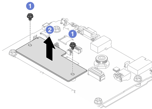
図 290. ファームウェアおよび RoT セキュリティー・モジュールの取り外し
