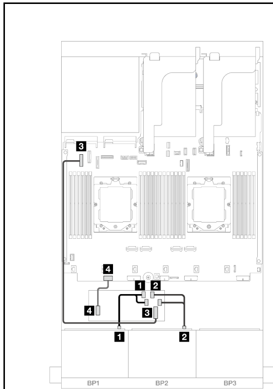
図 391. 2つのプロセッサが取り付けられた場合のケーブル配線
