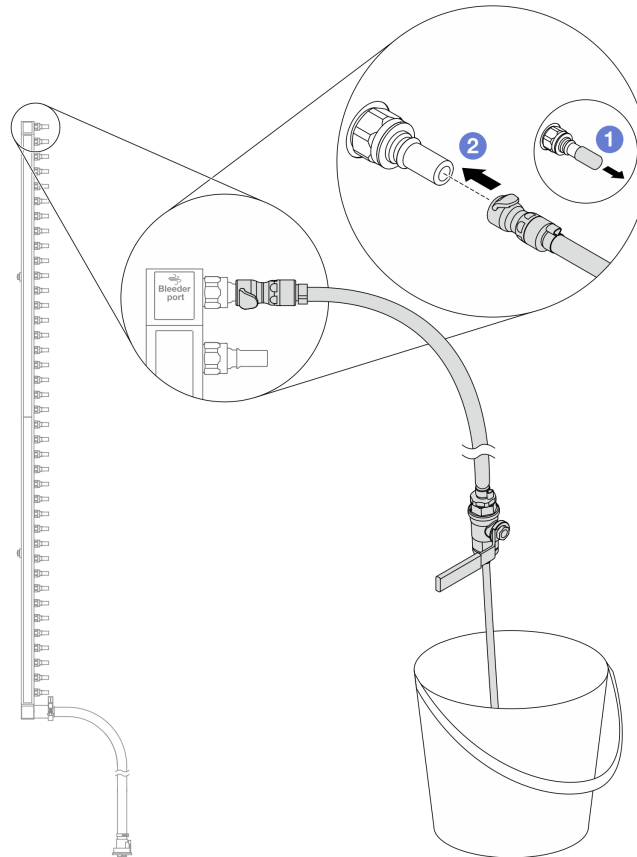
図 163. 供給側へのブリーダー・キットの取り付け
