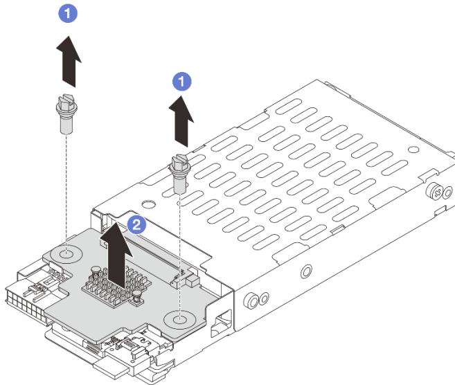
図 235. 7mm ドライブ・バックプレーンの取り外し (上部)
