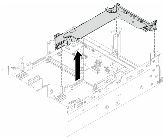
図 303. ライザー・ブラケットの取り外し
