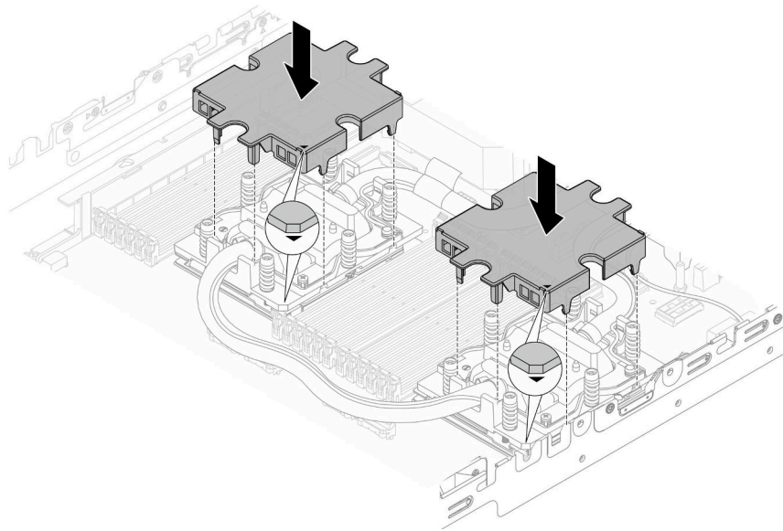
図109. コールド・プレート・カバーの取り付け
