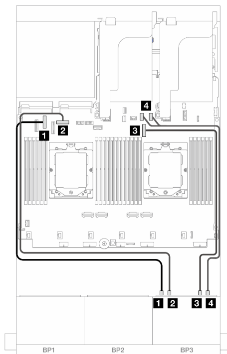
図 507. NVMe ケーブル配線
