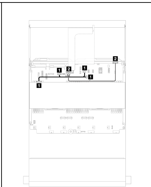
図 564. 中央/背面バックプレーン電源ケーブル配線
