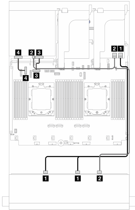
図 555. 2つのプロセッサが取り付けられた場合のケーブル配線
