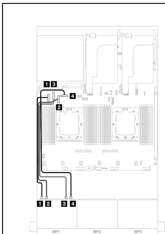
図 384. 2つのプロセッサが取り付けられた場合のケーブル配線
