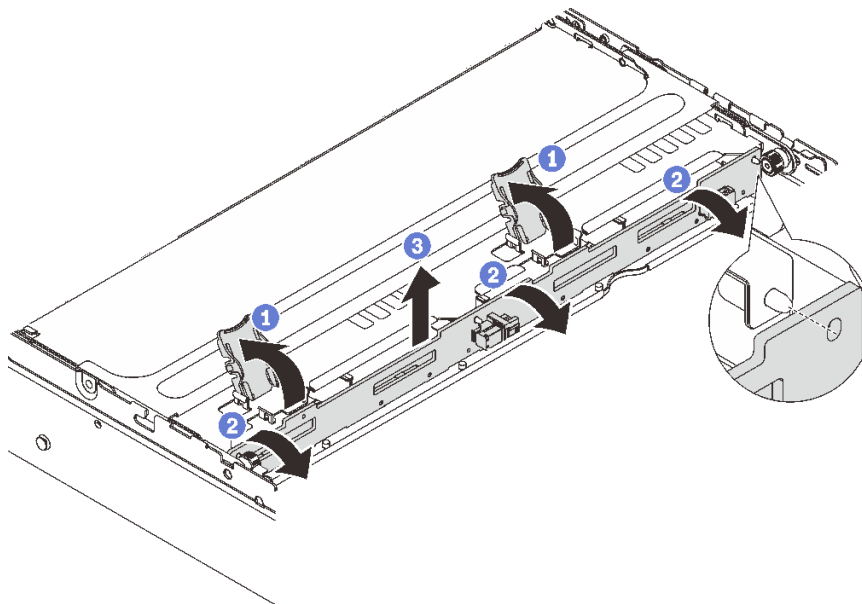
図185. 中央 3.5 型ドライブ・バックプレーンの取り外し
