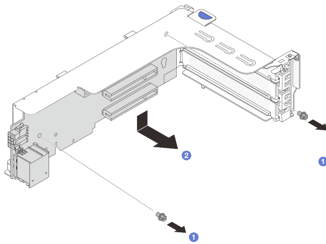
図 271. ライザー 1 ケージまたはライザー 2 ケージからのライザー・カードの取り外し
