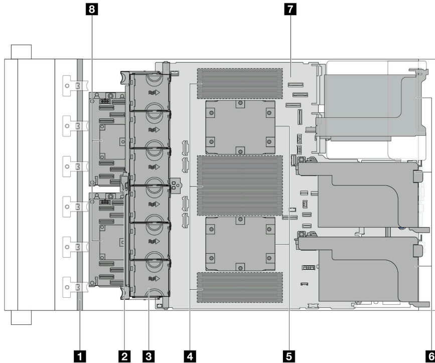
图 9. 带有标准散热器的俯视图
