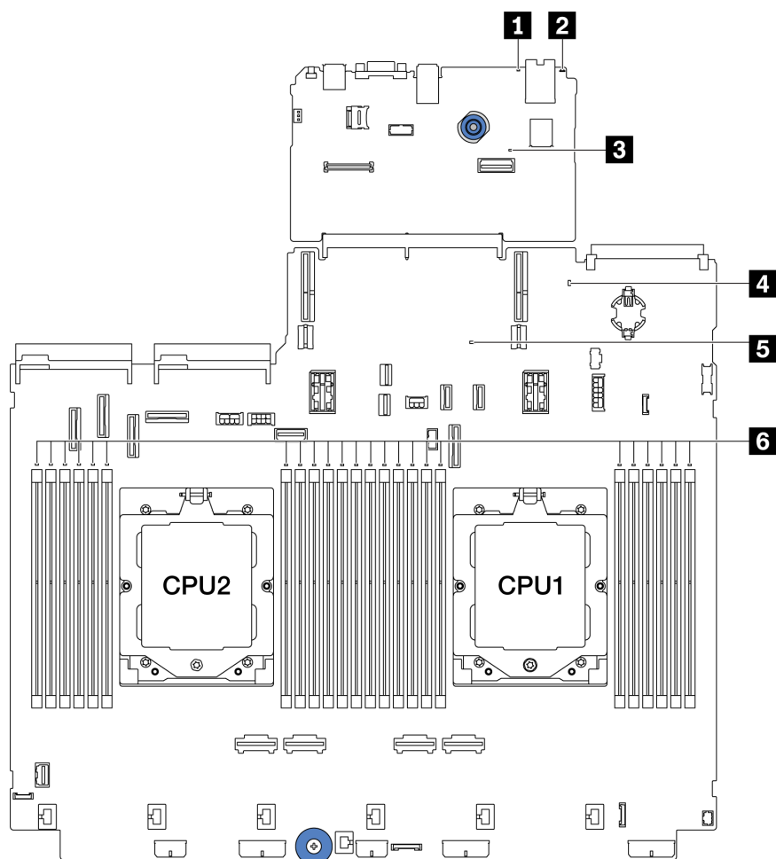
图 19. 主板组合件 LED
