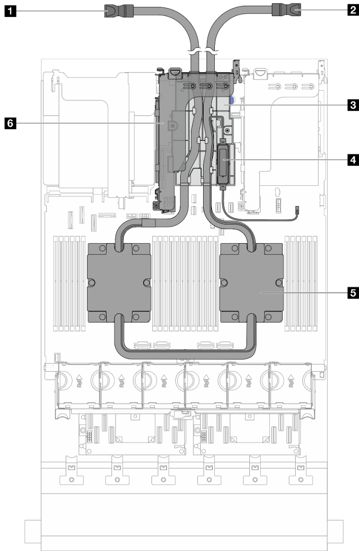
图 10. 带有 DWCM 的服务器型号的俯视图
