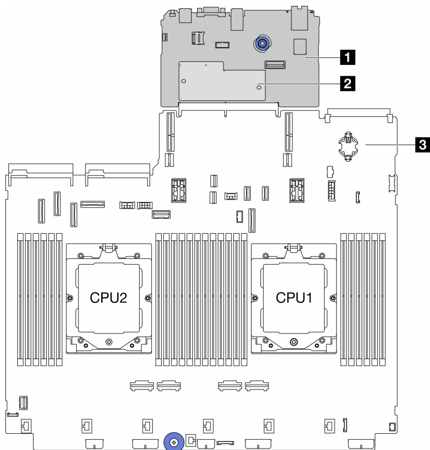
图 11. 主板组合件布局
