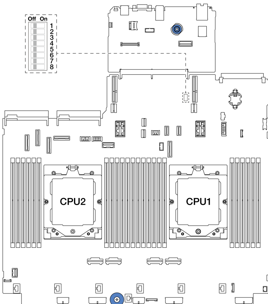
图 13. 主板组合件上的开关组
