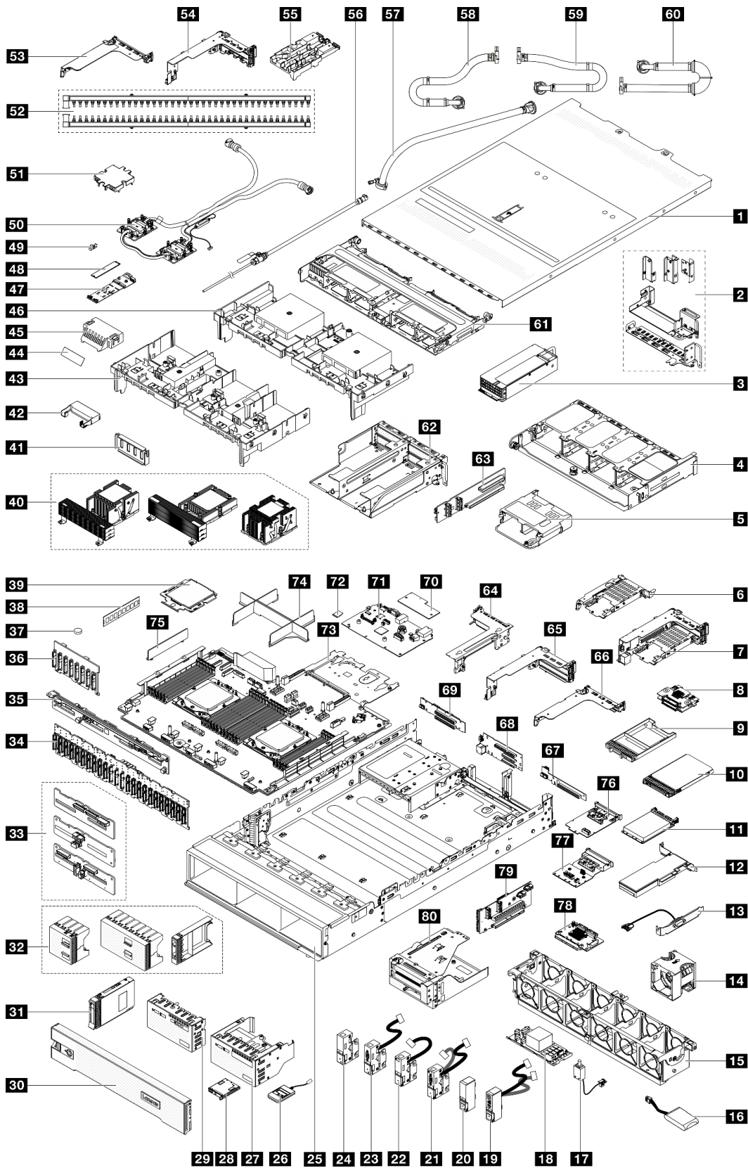
图 21. 服务器组件 (2.5 英寸硬盘插槽机箱)
