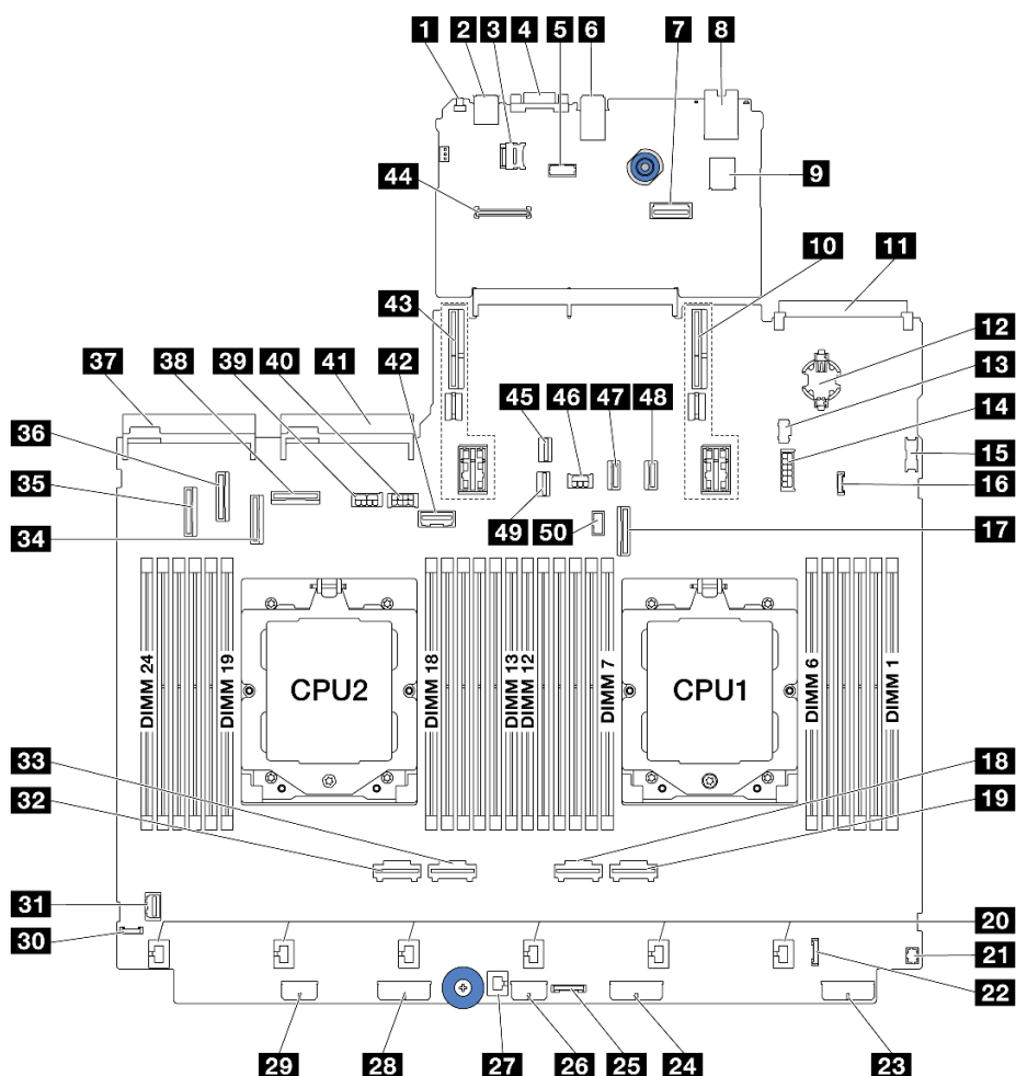
图 12. 主板组合件接口
