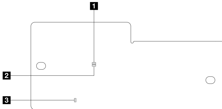
图 20. 固件和 RoT 安全模块上的 LED
