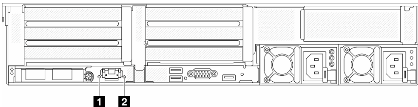
图 16. 背面系统 LED
