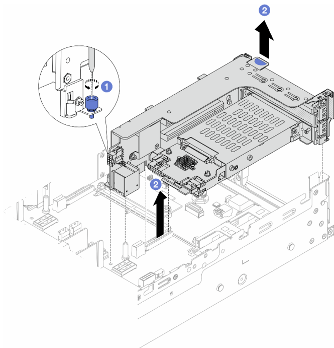
图 232. 卸下 2FH + 7 毫米固态硬盘转接卡架
