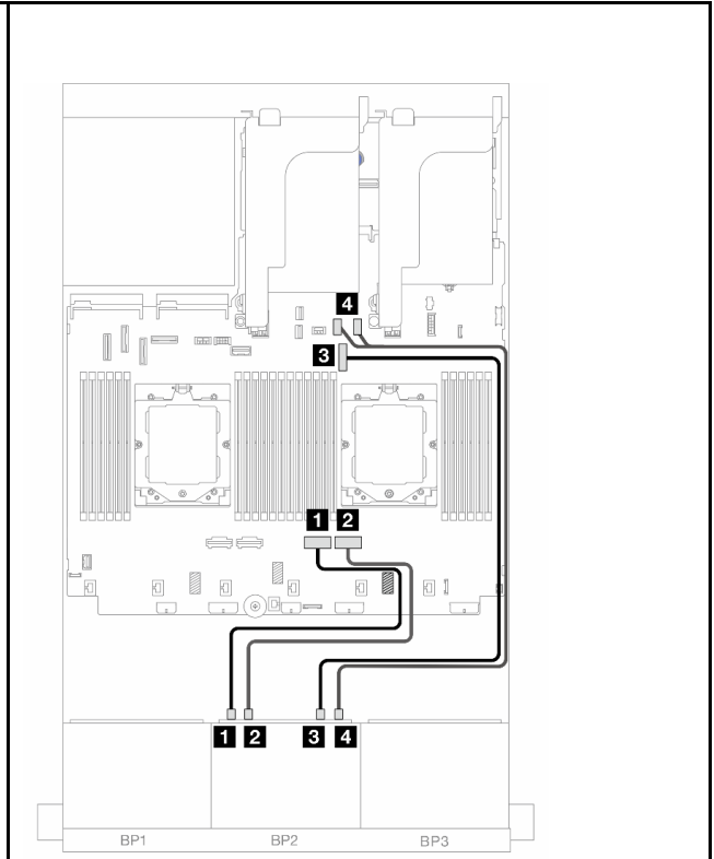
图 408. 装有一个处理器时的线缆布放
