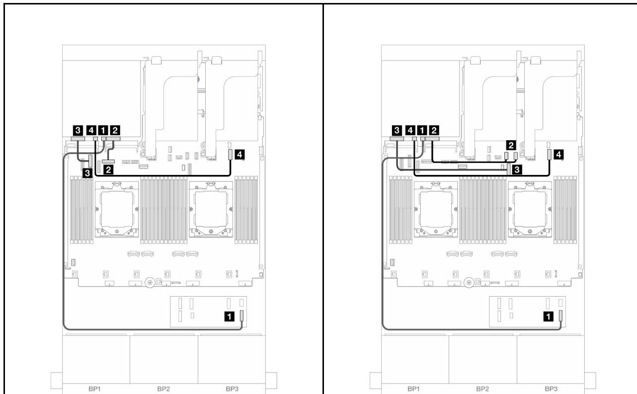
图 455. 装有两个处理器时的线缆布放
