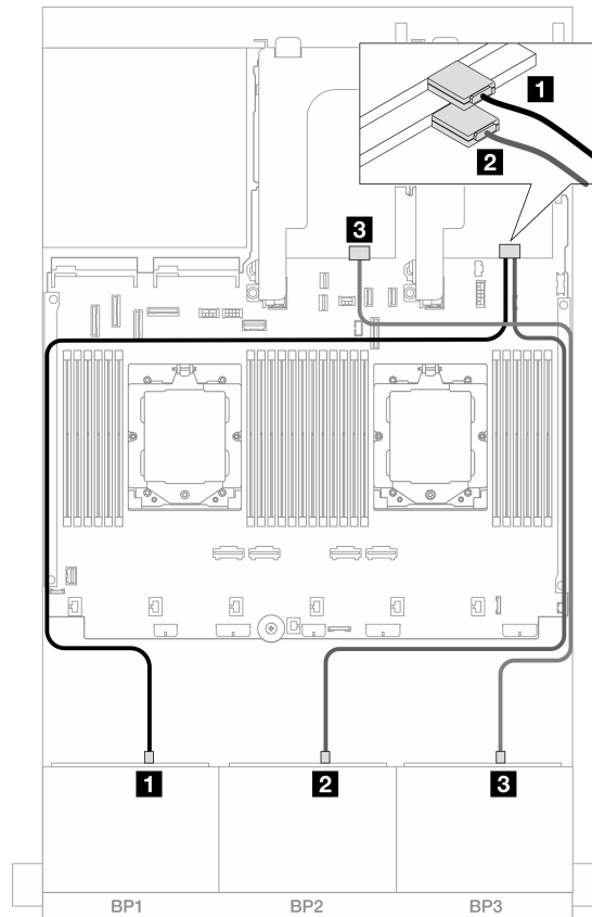
图 489. 到 8i 三模式适配器的 SAS/SATA 线缆布放
