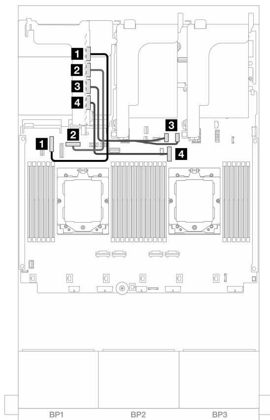
图 352. x16/x16 Gen 5 PCIe 转接卡 3 的信号线缆连接
