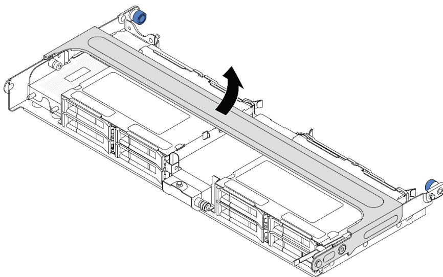
图 221. 打开中间硬盘仓的手柄
