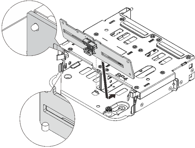
图 245. 安装 4 x 2.5 英寸背面硬盘背板
