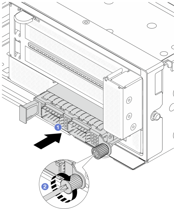
图 51. 安装正面 OCP 模块
