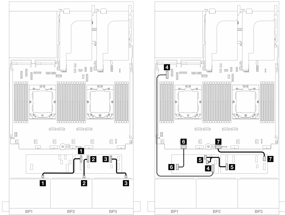
图 466. 到 CFF 扩展器和 CFF 16i 适配器的 SAS/SATA 线缆布放
