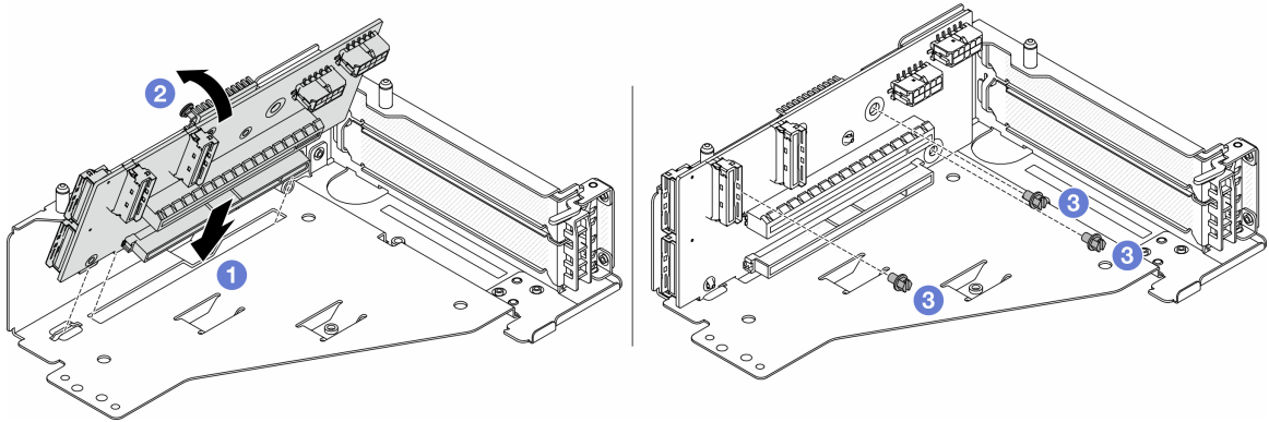
图 66. 安装转接卡
