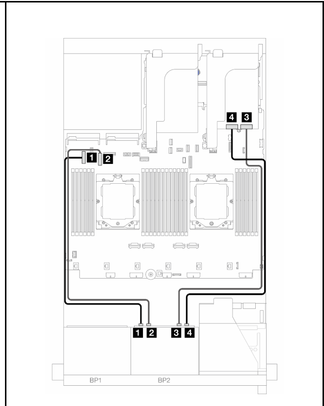
图 421. NVMe 线缆布放
