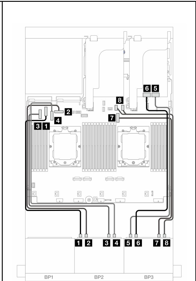
图 502. NVMe 线缆布放
