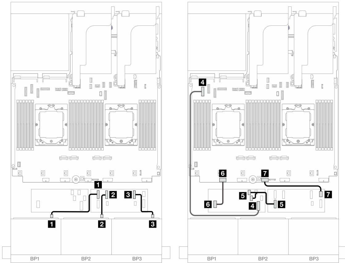
图 481. 到 CFF 扩展器和 CFF 16i 适配器的 SAS/SATA 线缆布放
