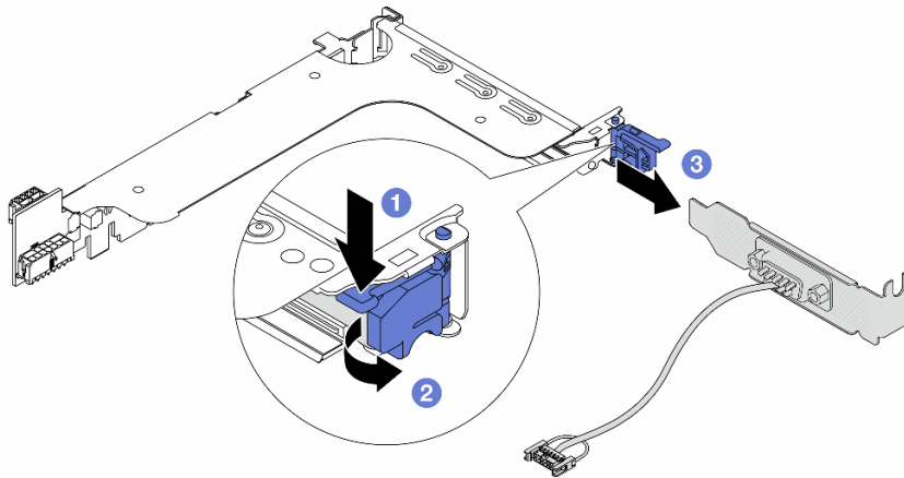
图 304. 卸下串口模块
