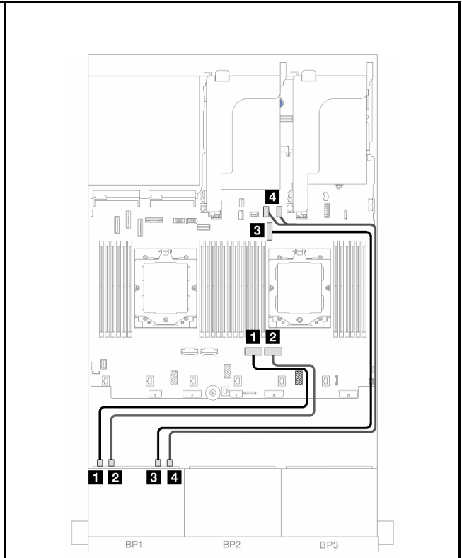
图 367. 装有一个处理器时的线缆布放
