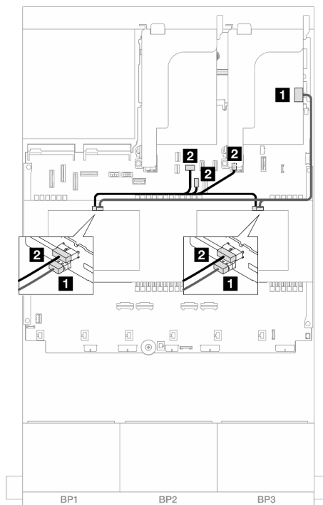
图 474. 中间背板线缆布放
