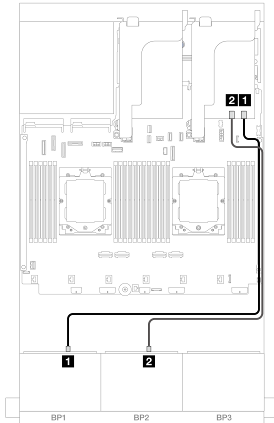
图 403. 到三模式 16i 适配器的信号线缆布放
