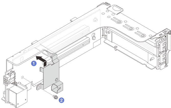
图 239. 安装 7 毫米硬盘仓固定夹
