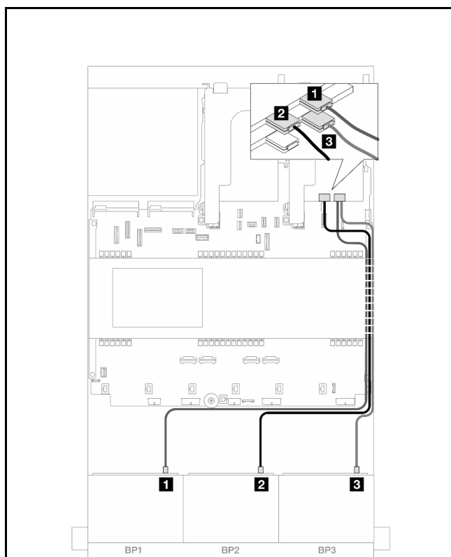
图 459. 正面背板线缆布放
