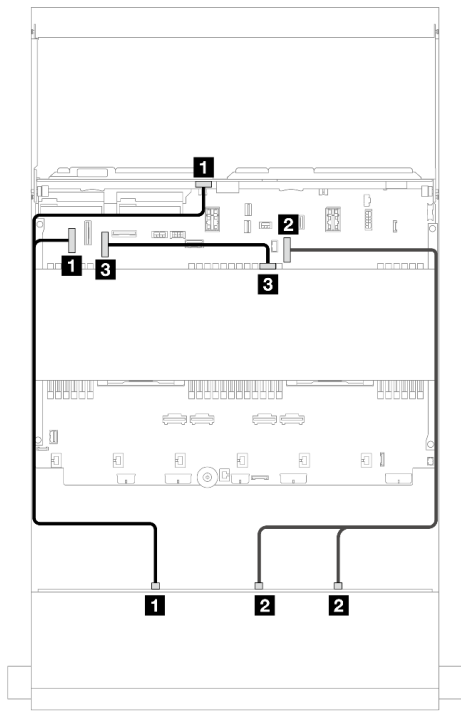
图 563. 正面/中间/背面背板信号线缆布放
