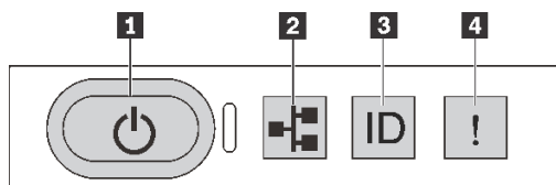
图 590. 正面操作员面板 LED
