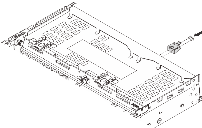
图 259. 安装顶盖支架
