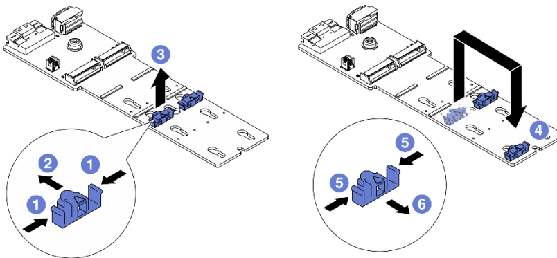
图 115. 调整 M.2 固定器
