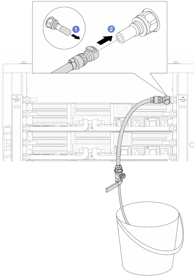
图 157. 将排气套件安装到回流侧
