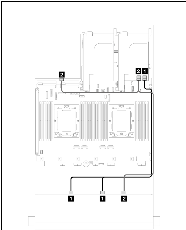
图 553. 正面/背面背板信号线缆布放
