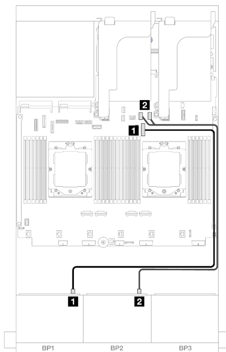
图 389. 装有一个处理器时的线缆布放
