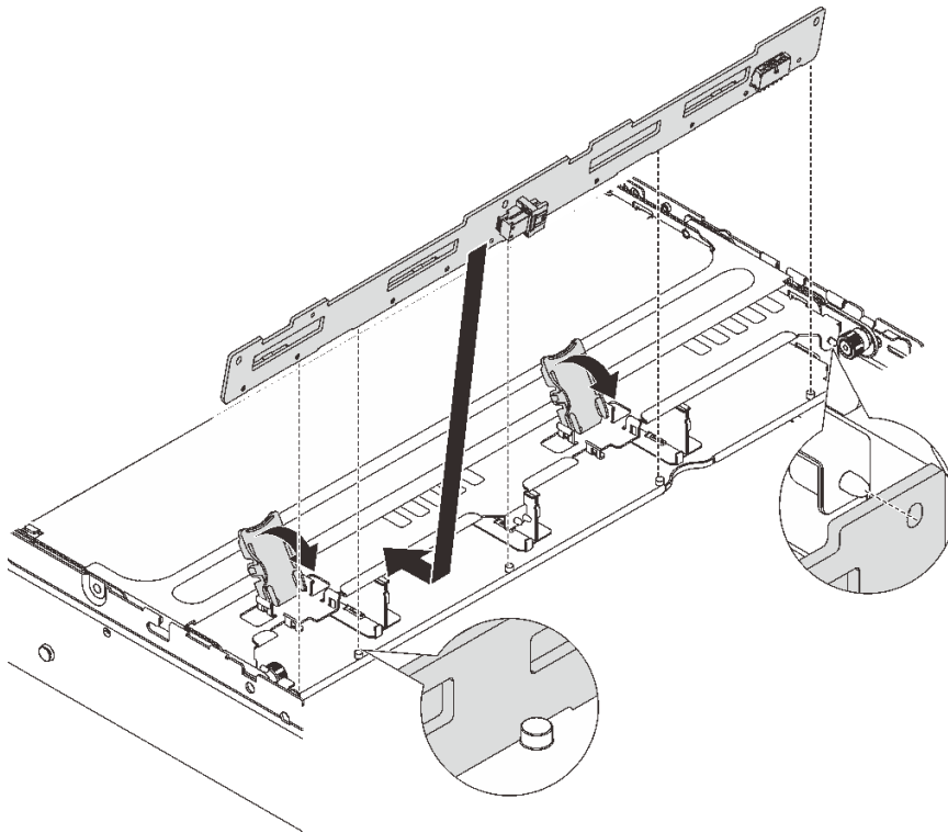
图 187. 安装 3.5 英寸中间硬盘背板
