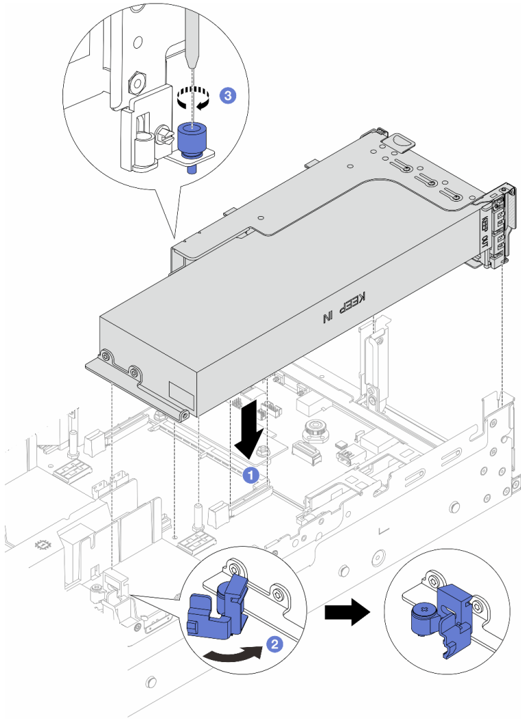
图 93. 安装带有 GPU 适配器的转接卡 1 组合件
