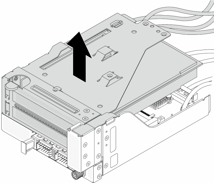
图 63. 提起转接卡 5 组合件
