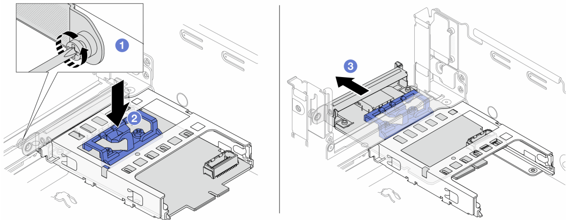
图 130. 卸下管理 NIC 适配器
