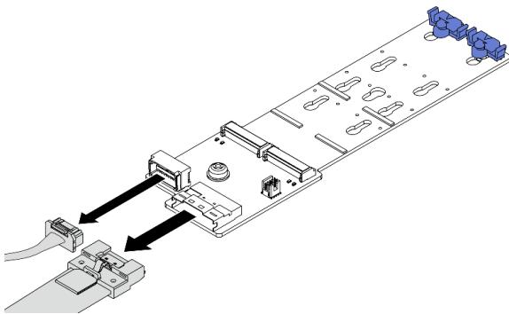
图 118. 从 M.2 x4 非 RAID SATA/NVMe 2 插槽背板上拔下线缆
