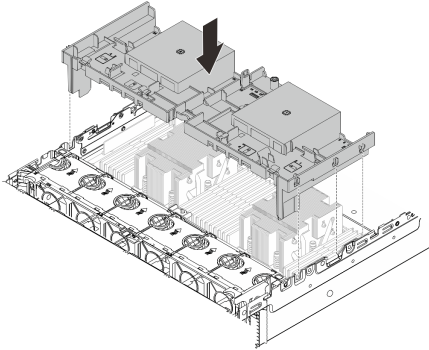
图 33. 安装导风罩
