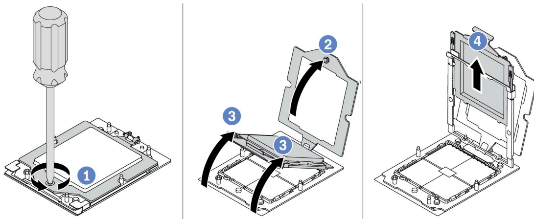
图 196. 卸下处理器
