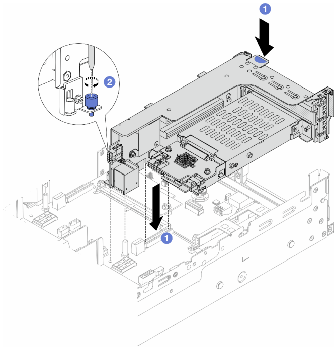
图 241. 安装 2FH + 7 毫米固态硬盘转接卡架
