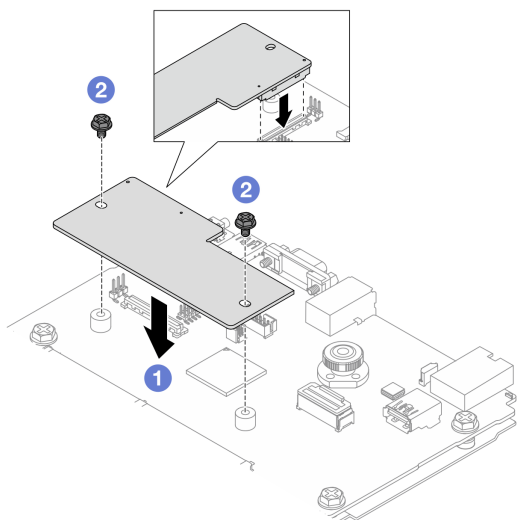
图 291. 安装固件和 RoT 安全模块
