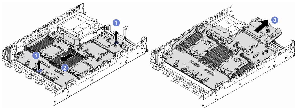
图 292. 卸下主板组合件
