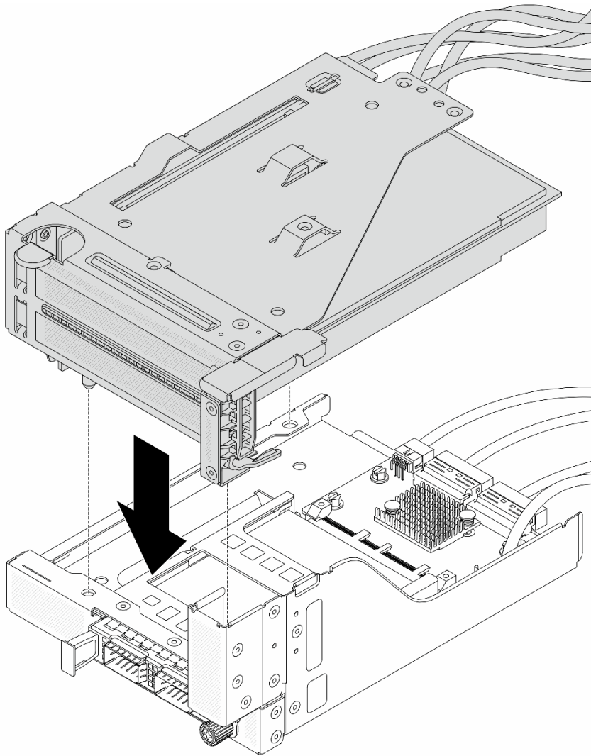
图 68. 将转接卡 5 组合件安装到正面 OCP 组合件上
