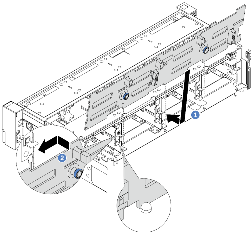
图 76. 安装 3.5 英寸硬盘背板
