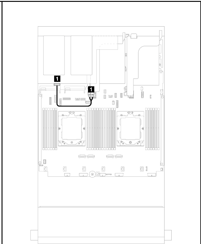
图 552. 背面背板电源线布放
