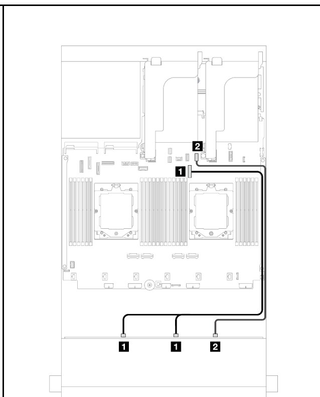
图 548. 装有一个处理器时的线缆布放
