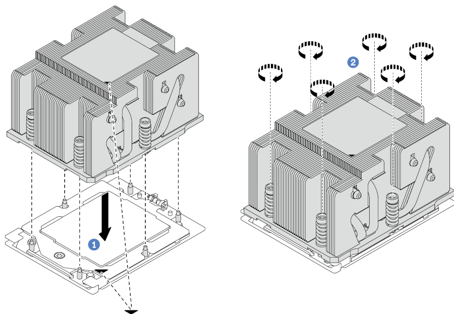
图 201. 安装标准散热器
