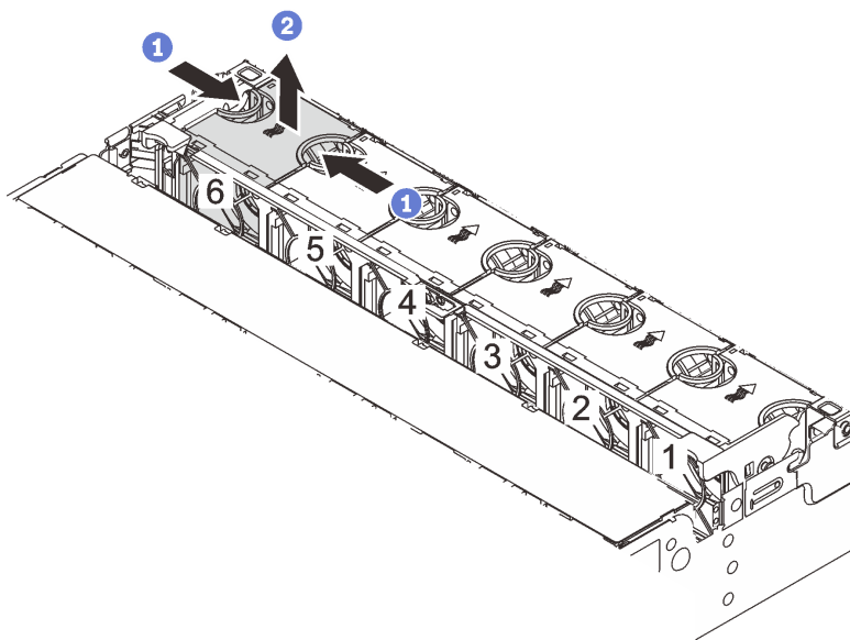
图 298. 卸下系统风扇
