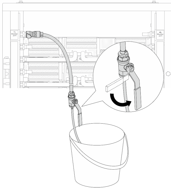
图 177. 打开供给侧的泄放阀门
