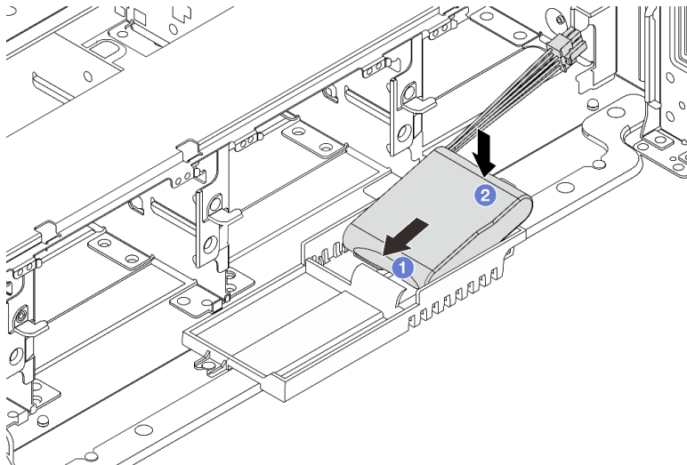
图 217. 将 RAID 快速充电模块安装到超级电容器夹持器上
