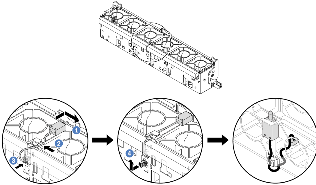
图 100. 安装入侵感应开关
