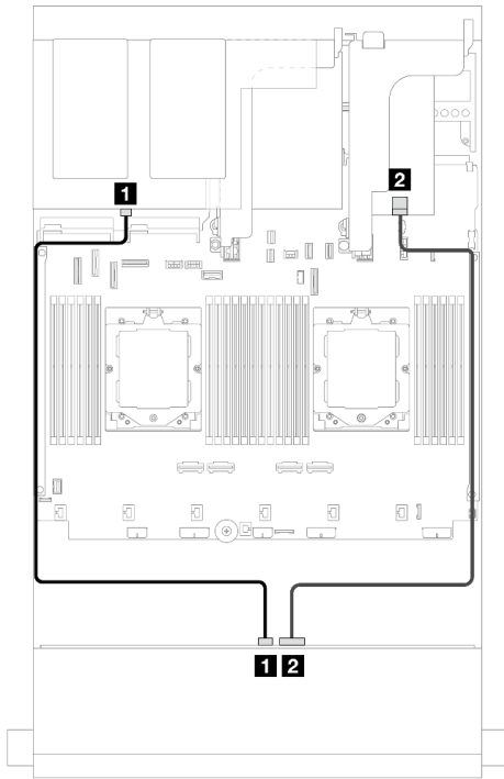
图 580. 正面/背面背板信号线缆布放
