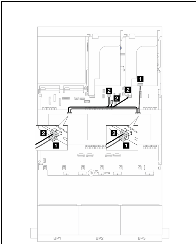
图 400. 中间背板线缆布放
