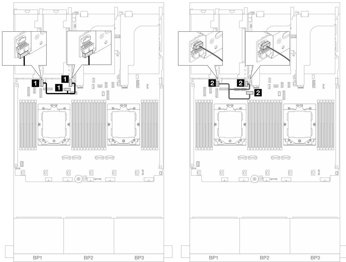
图 353. 转接卡 3/4 电源线和边带线缆布放
