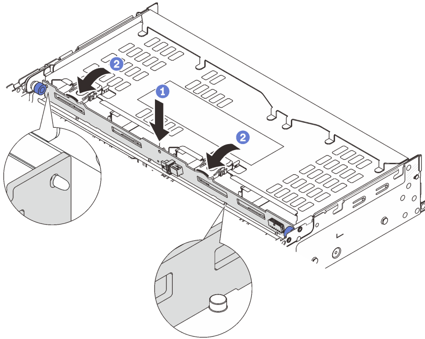
图 257. 安装 4 x 3.5 英寸背面硬盘背板
