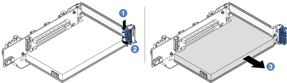
图 269. 从转接卡 3 组合件上卸下 PCIe 适配器
