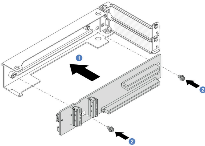
图 276. 将转接卡安装到 4LP 转接卡 3/4 架上
