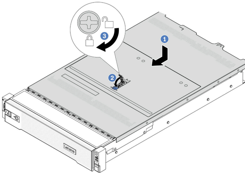
图 310. 安装顶盖
