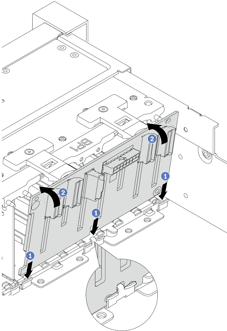
图 73. 安装 8 插槽硬盘背板
