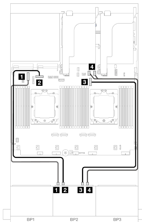
图 413. NVMe 线缆布放
