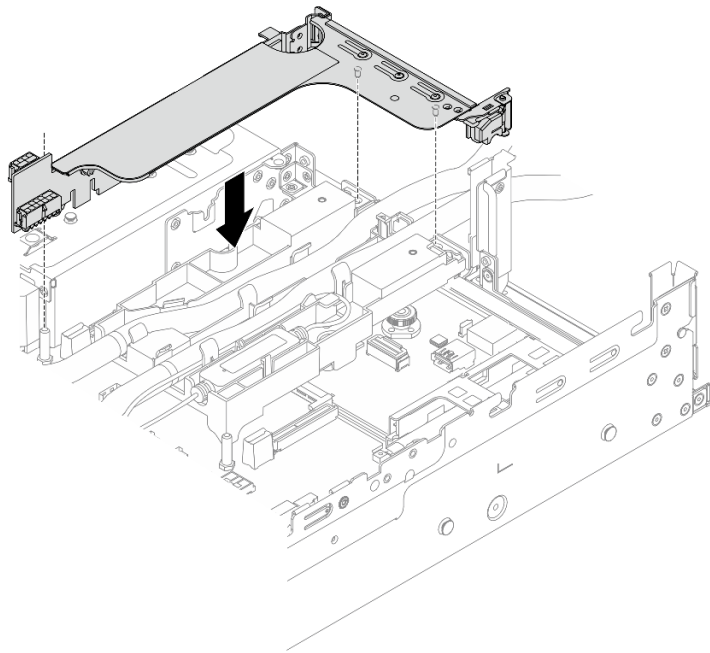
图 112. 安装 1FH 转接卡架
