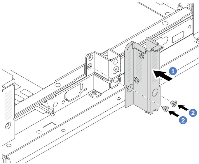
图 230. 安装 B1 背面壁挂支架（中间）
