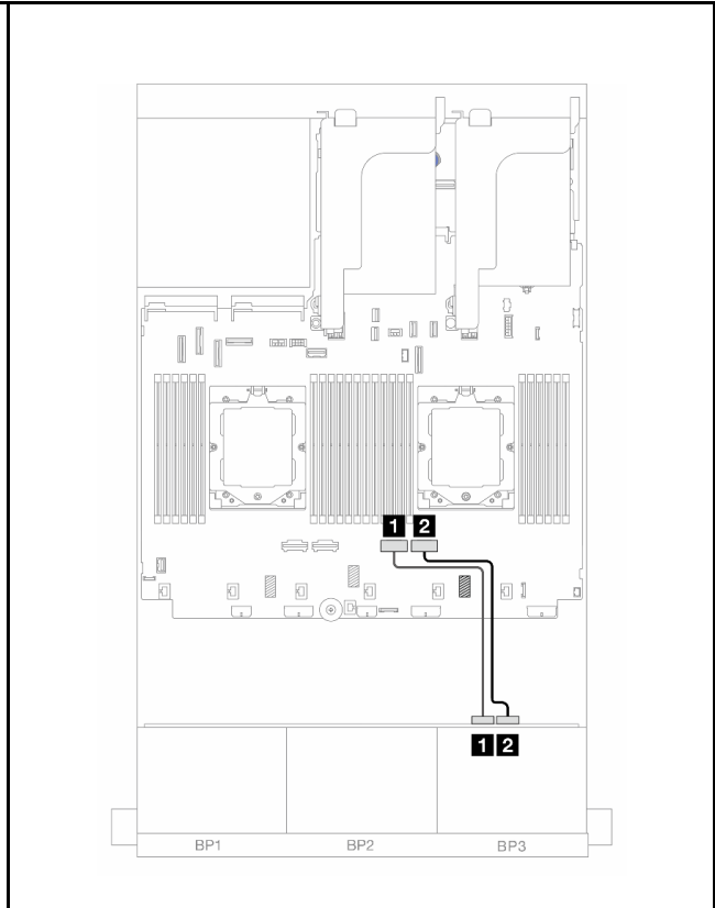
图 570. NVMe 线缆布放
