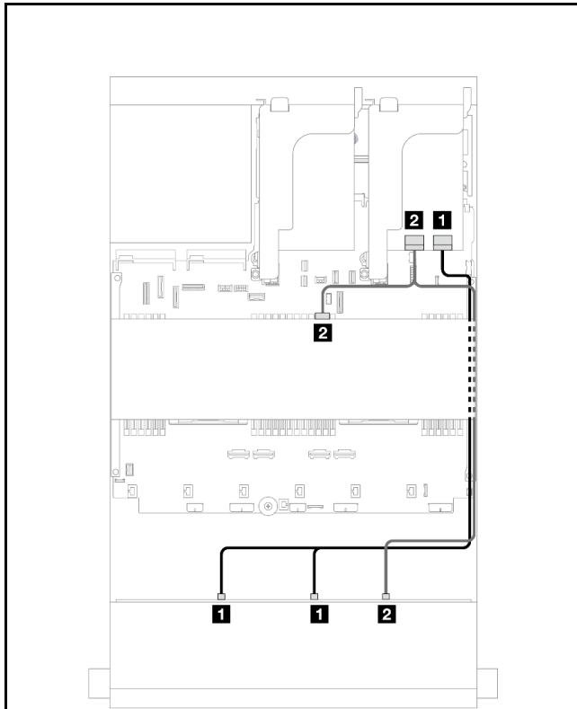
图 558. 正面/中间背板信号线缆布放
