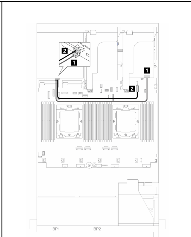
图 401. 背面背板线缆布放
