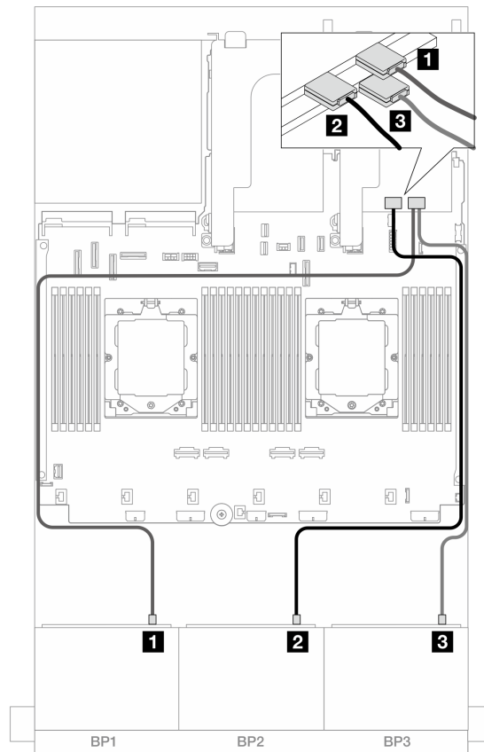
图 439. 到 8i/16i 适配器的 SAS/SATA 线缆布放
