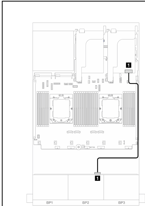
图 536. 正面背板线缆布放
