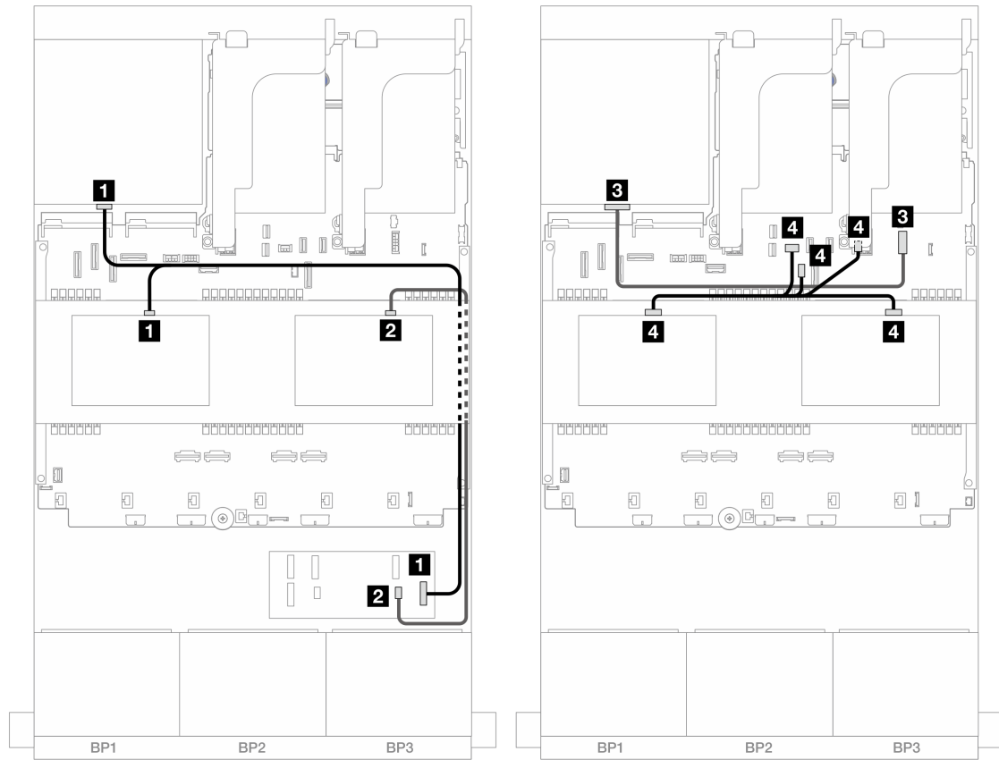
图 483. 中间/背面背板线缆布放
