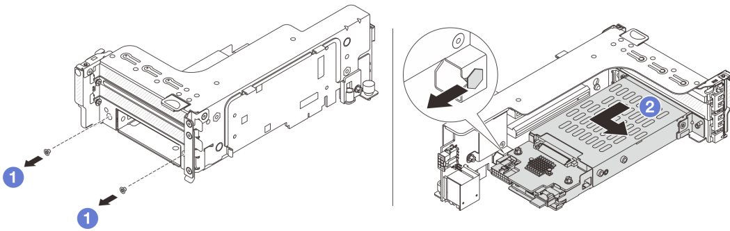
图 234. 从转接卡组合件上卸下 7 毫米硬盘仓
