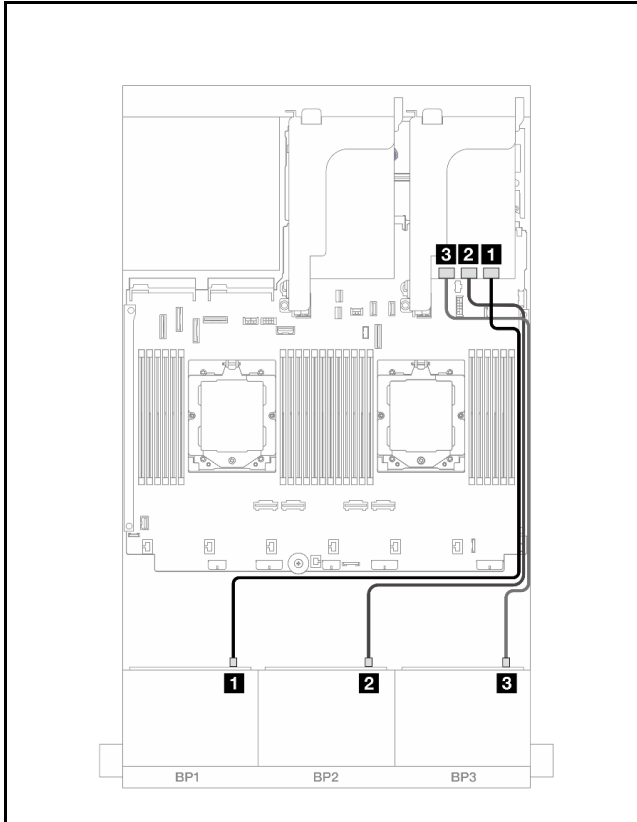
图 469. 正面背板线缆布放
