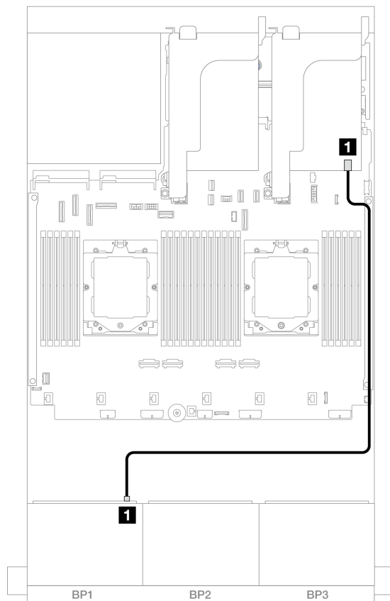
图 426. 到 8i 适配器的 SAS/SATA 线缆布放
