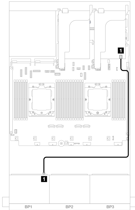
图 362. 到 8i/16i RAID/HBA 适配器的 SAS/SATA 线缆布放
