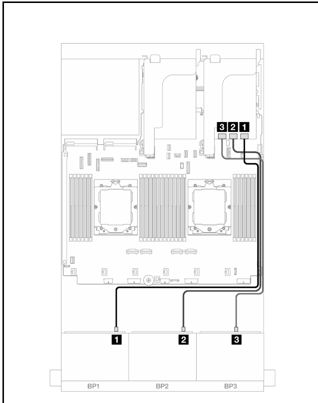
图 508. SAS/SATA 线缆布放
