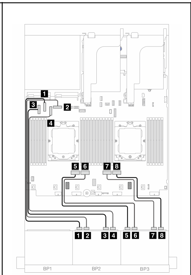
图 500. NVMe 线缆布放
