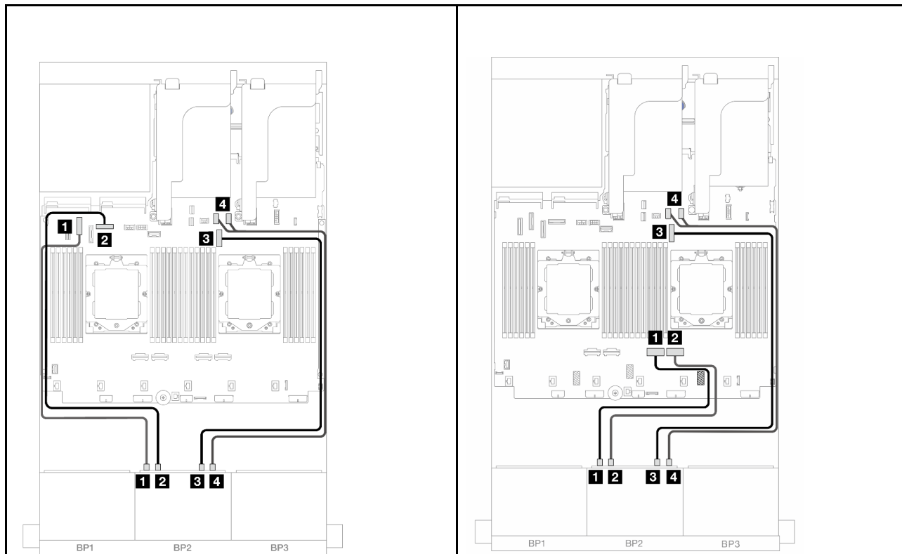
图 427. 装有两个处理器时的线缆布放
