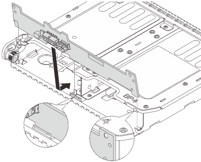
图 253. 安装 2 x 3.5 英寸背面硬盘背板
