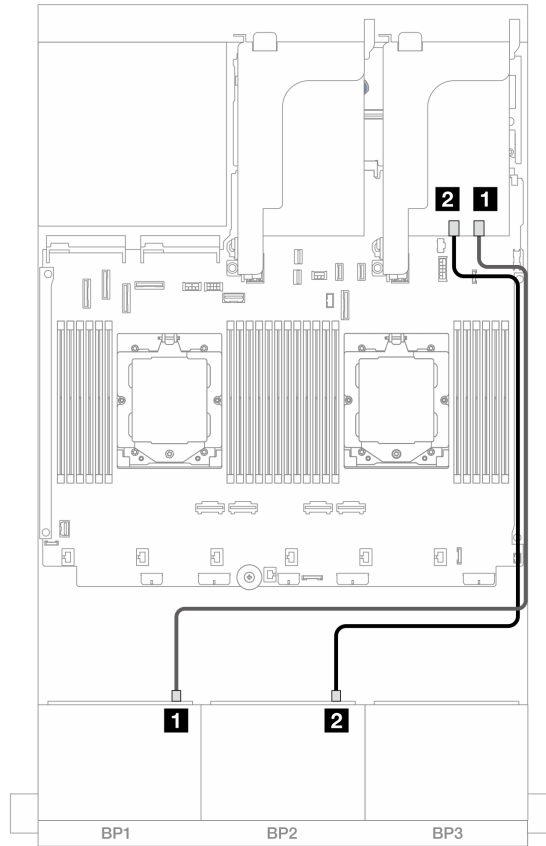
图 399. 到 16i RAID/HBA 适配器的 SAS/SATA 线缆布放
