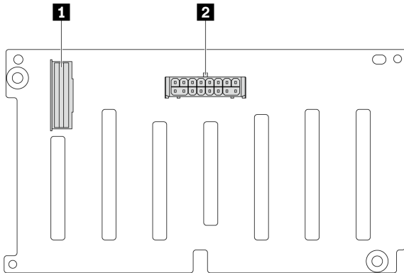
图 311. 8 x 2.5 英寸 SAS/SATA 背板接口
