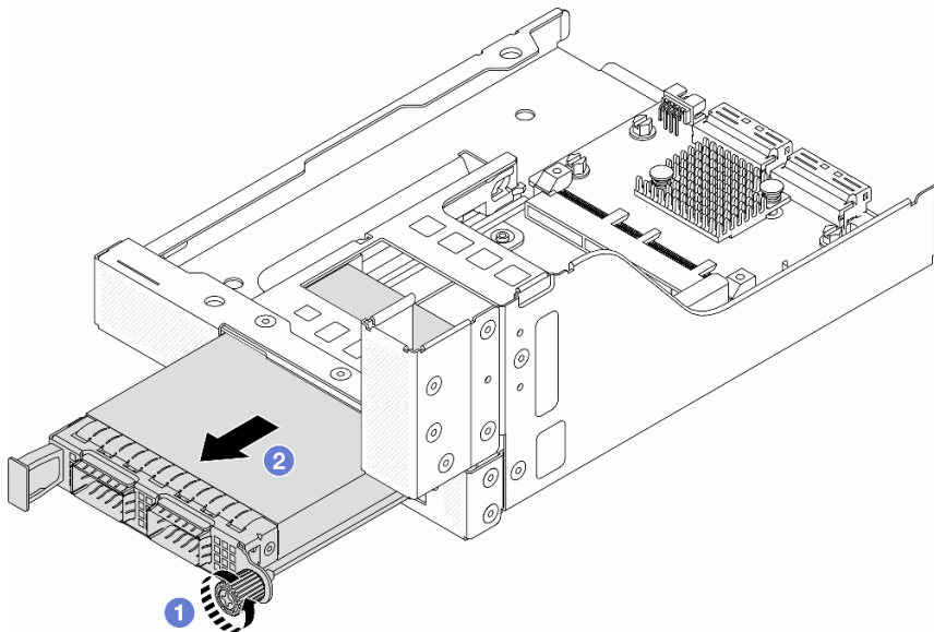
图 54. 卸下 OCP 模块
