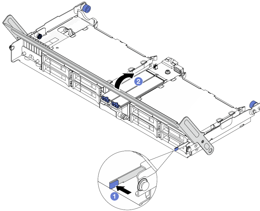
图 126. 合上中间硬盘仓的手柄
