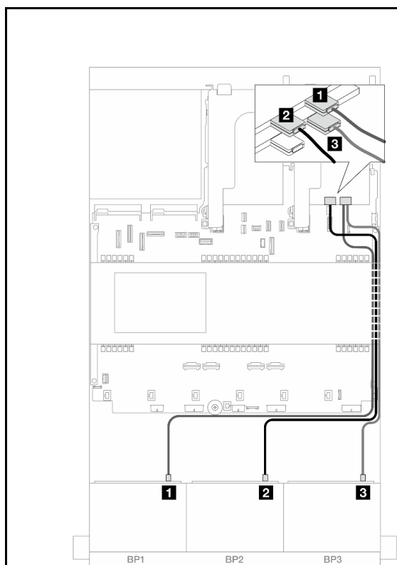
图 475. 正面背板线缆布放
