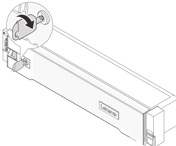
图 284. 解锁安全挡板
