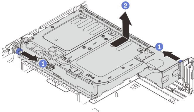
图 251. 卸下 2 x 3.5 英寸背面硬盘仓
