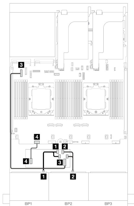
图 412. SAS/SATA 线缆布放
