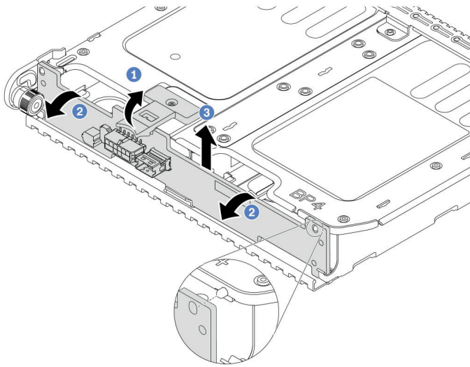
图 252. 卸下 2 x 3.5 英寸背面硬盘背板
