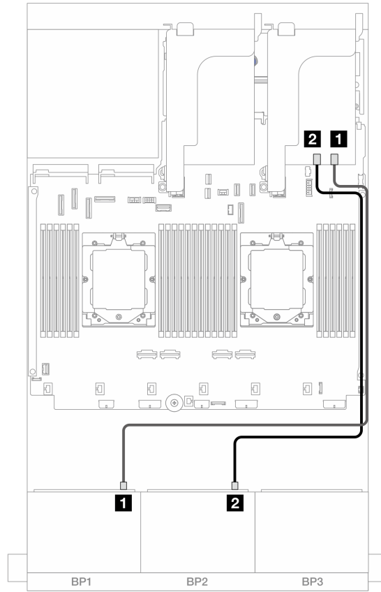
图 517. 到 16i RAID/HBA 适配器的 SAS/SATA 线缆布放
