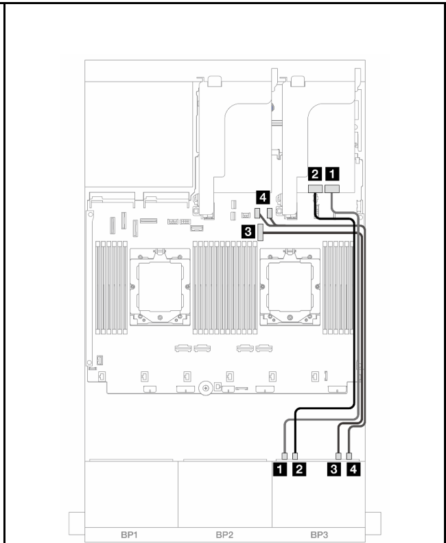
图 511. NVMe 线缆布放
