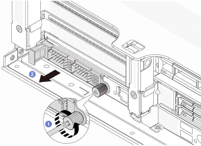
图 260. 卸下背面 OCP 模块
