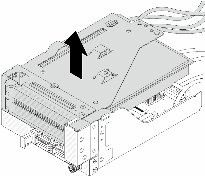
图 53. 提起转接卡 5 组合件
