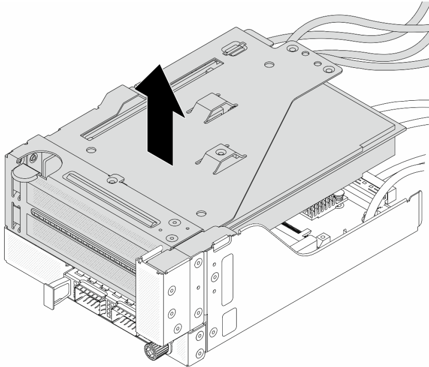
图 39. 提起转接卡 5 组合件
