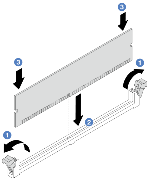
图 180. 安装内存条
