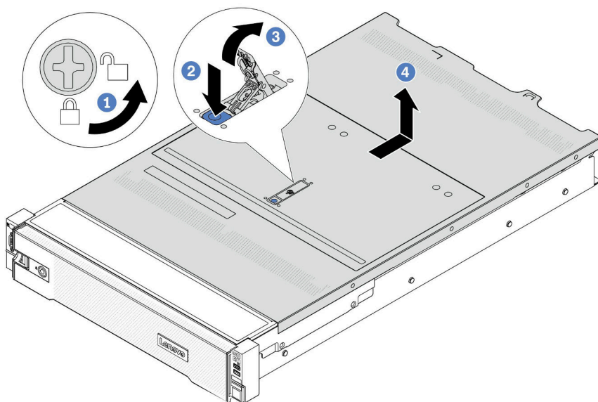
图 309. 卸下顶盖
