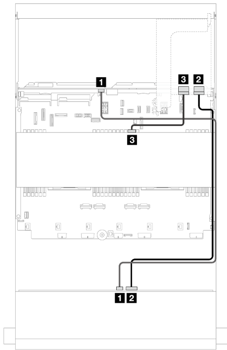
图 585. 背板信号线缆布放
