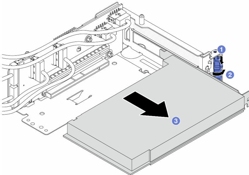
图 40. 从转接卡 5 架上卸下 PCIe 适配器
