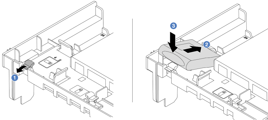
图 219. 将 RAID 快速充电模块安装到导风罩上
