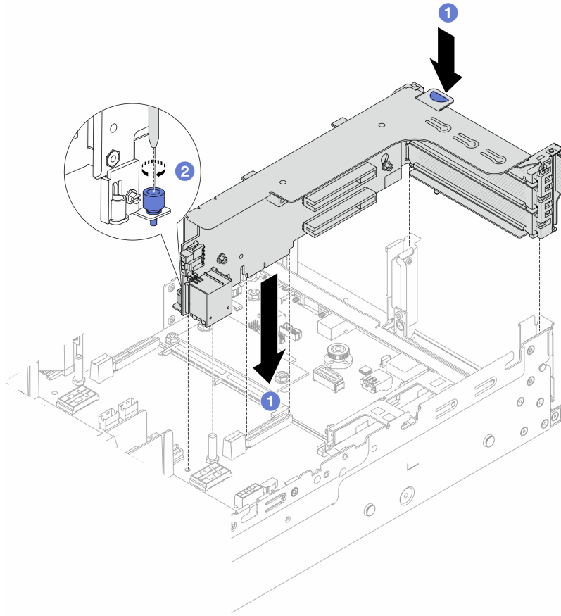
图 280. 安装转接卡 1 组合件
