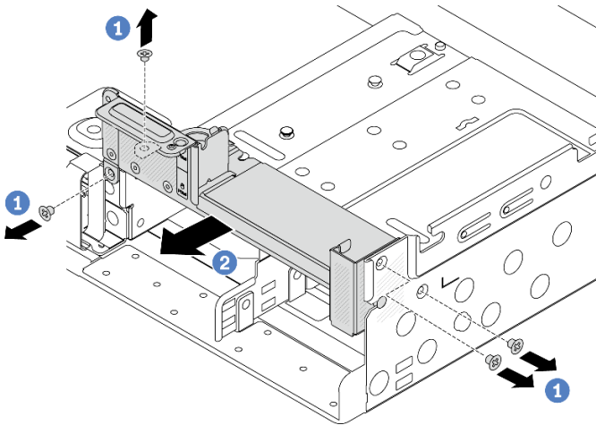
图 228. 卸下 C1 背面壁挂支架（右侧）
