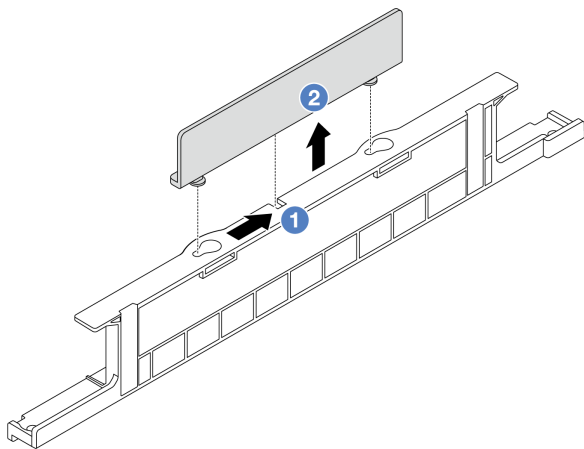
图 34. 卸下 2U 线缆壁挂支架
