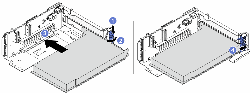
图 67. 将 PCIe 适配器安装到转接卡 5 架上
