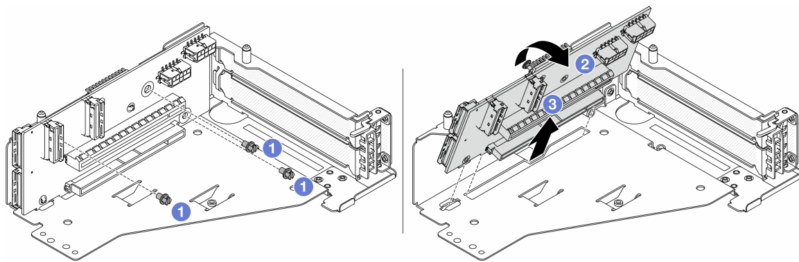
图 65. 从转接卡 5 架上卸下转接卡
