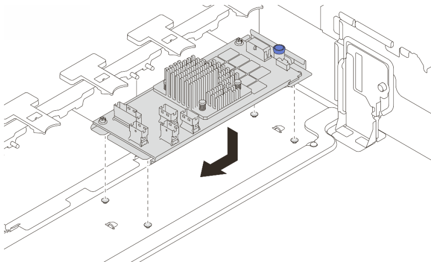
图 97. 安装内部 CFF 适配器
