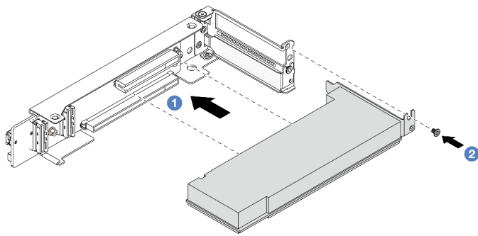
图 279. 将 PCIe 适配器安装到 4LP 转接卡 3/4 组合件上
