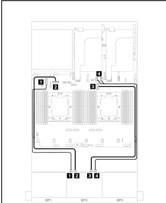
图 407. 装有两个处理器时的线缆布放
