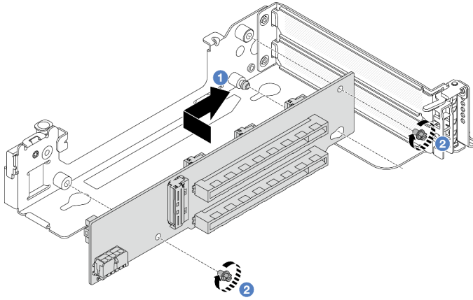
图 275. 将转接卡安装到转接卡 3 架上
