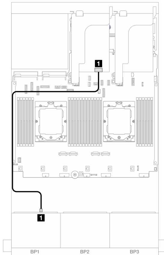
图 497. 到 8i 适配器的 SAS/SATA 线缆布放
