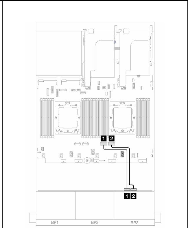
图 578. NVMe 线缆布放
