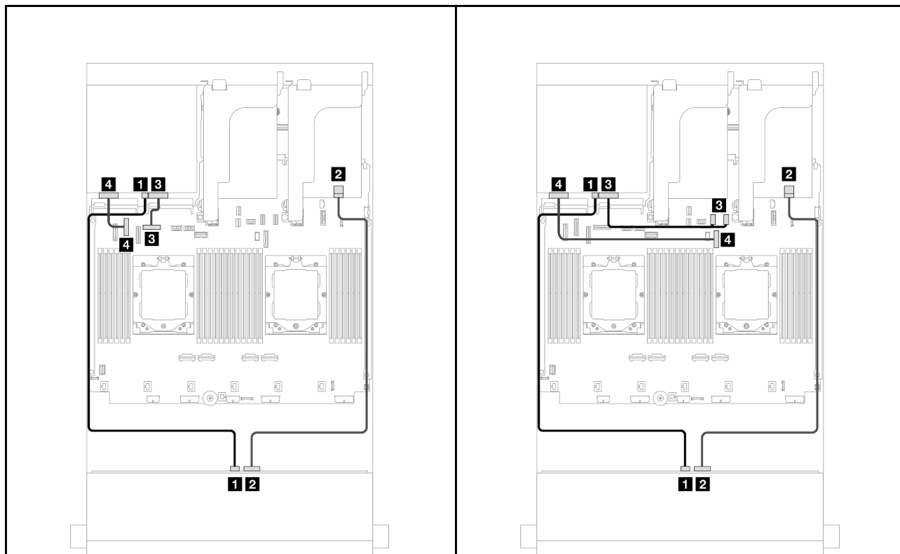
图 582. 装有两个处理器时的线缆布放
