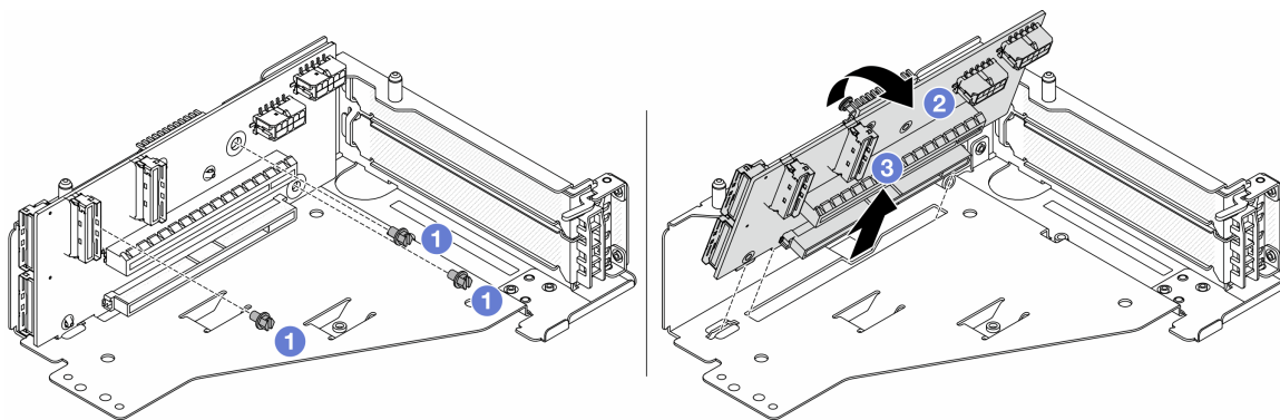
图 41. 从转接卡 5 架上卸下转接卡
