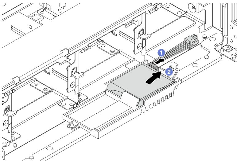
图 214. 从超级电容器夹持器上卸下 RAID 快速充电模块
