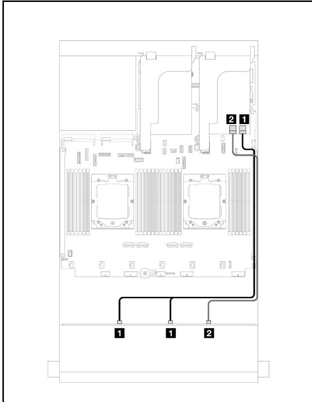
图 569. SAS/SATA 线缆布放
