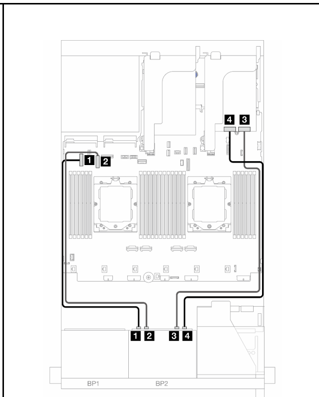
图 419. NVMe 线缆布放
