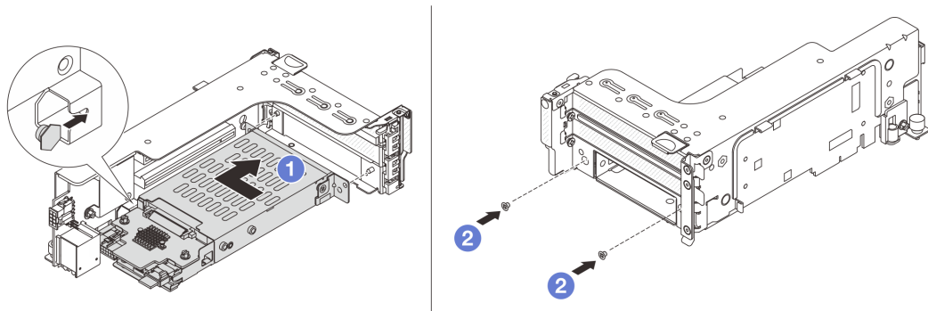
图 240. 将 7 毫米硬盘仓安装到转接卡组合件上
