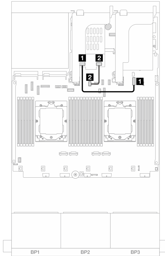
图 328. 7 毫米 RAID SATA/NVMe 2 插槽背板的线缆布放
