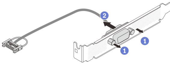
图 305. 拆卸串口模块
