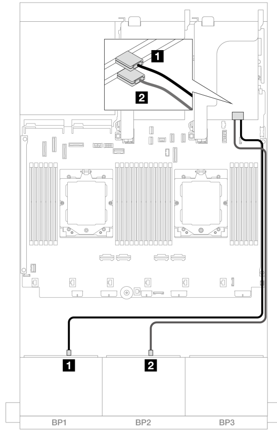
图 402. 到三模式 8i 适配器的信号线缆布放
