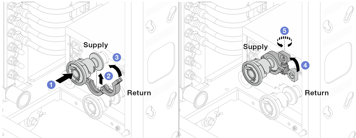
图 148. 安装球阀
