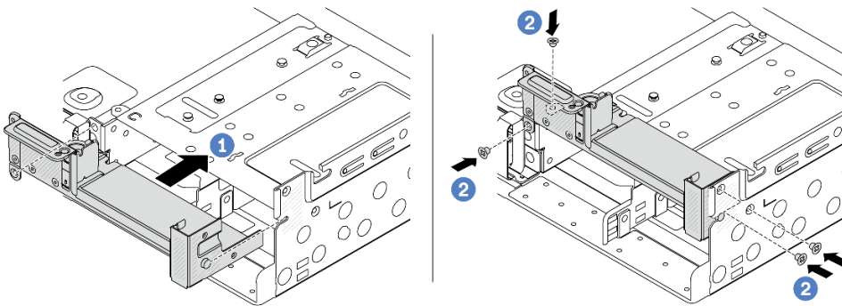
图 231. 安装 C1 背面壁挂支架（右侧）
