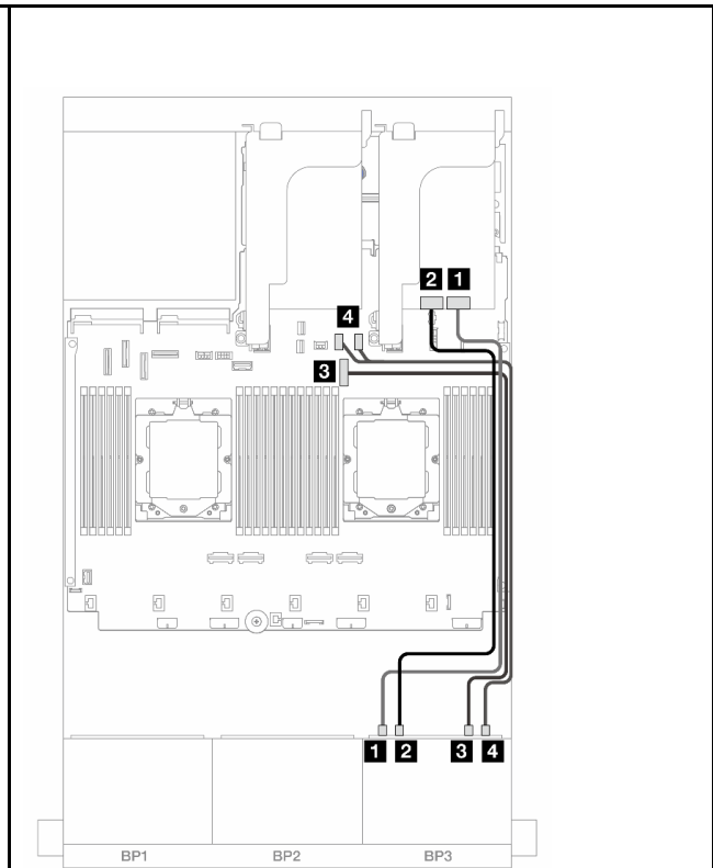
图 525. NVMe 线缆布局
