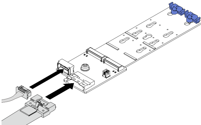
图 127. 将 M.2 线缆连接到 M.2 x4 非 RAID SATA/NVMe 2 插槽背板
