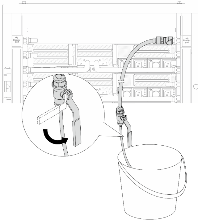
图 176. 打开回流侧的泄放阀门
