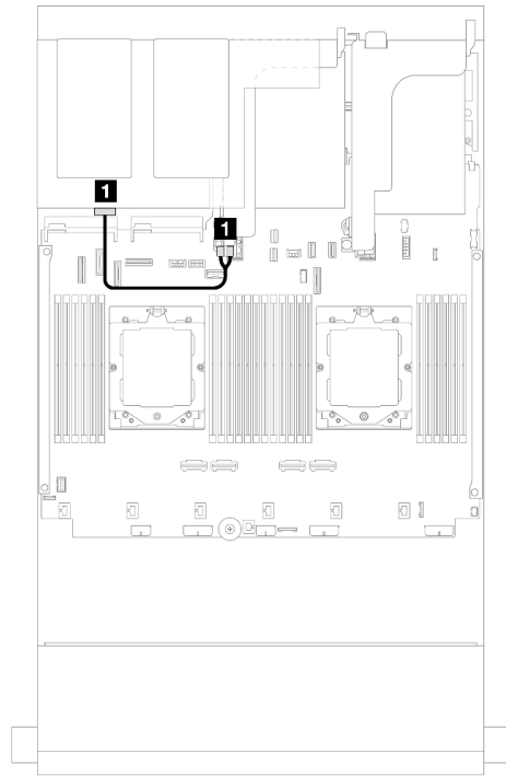
图 581. 背面背板电源线布放
