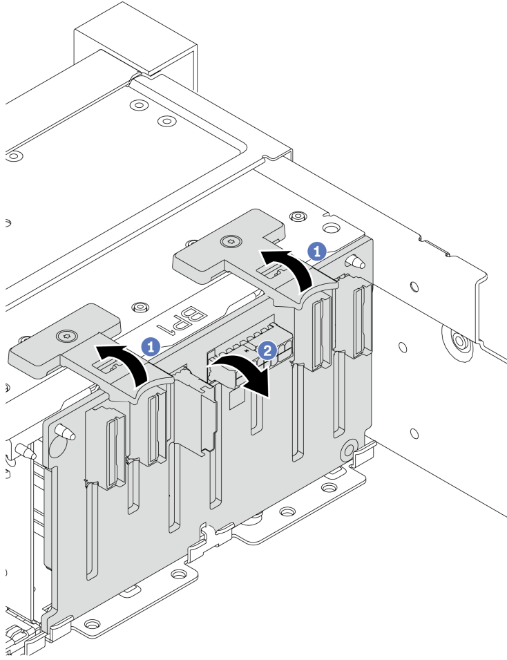
图 70. 卸下 8 插槽硬盘背板
