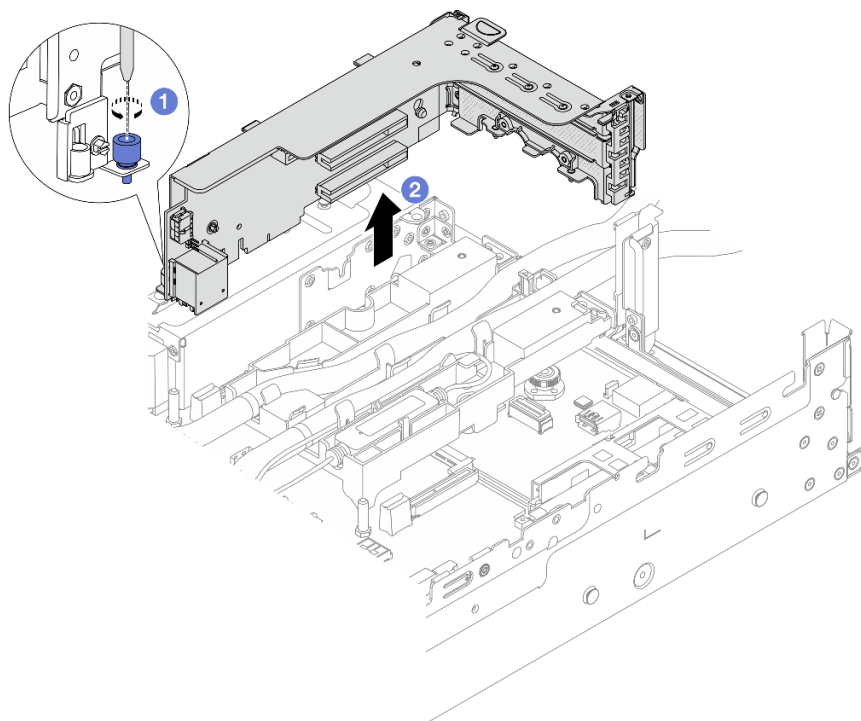
图 102. 卸下 3FH 转接卡架
