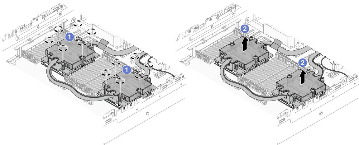
图 104. 卸下 DWCM
