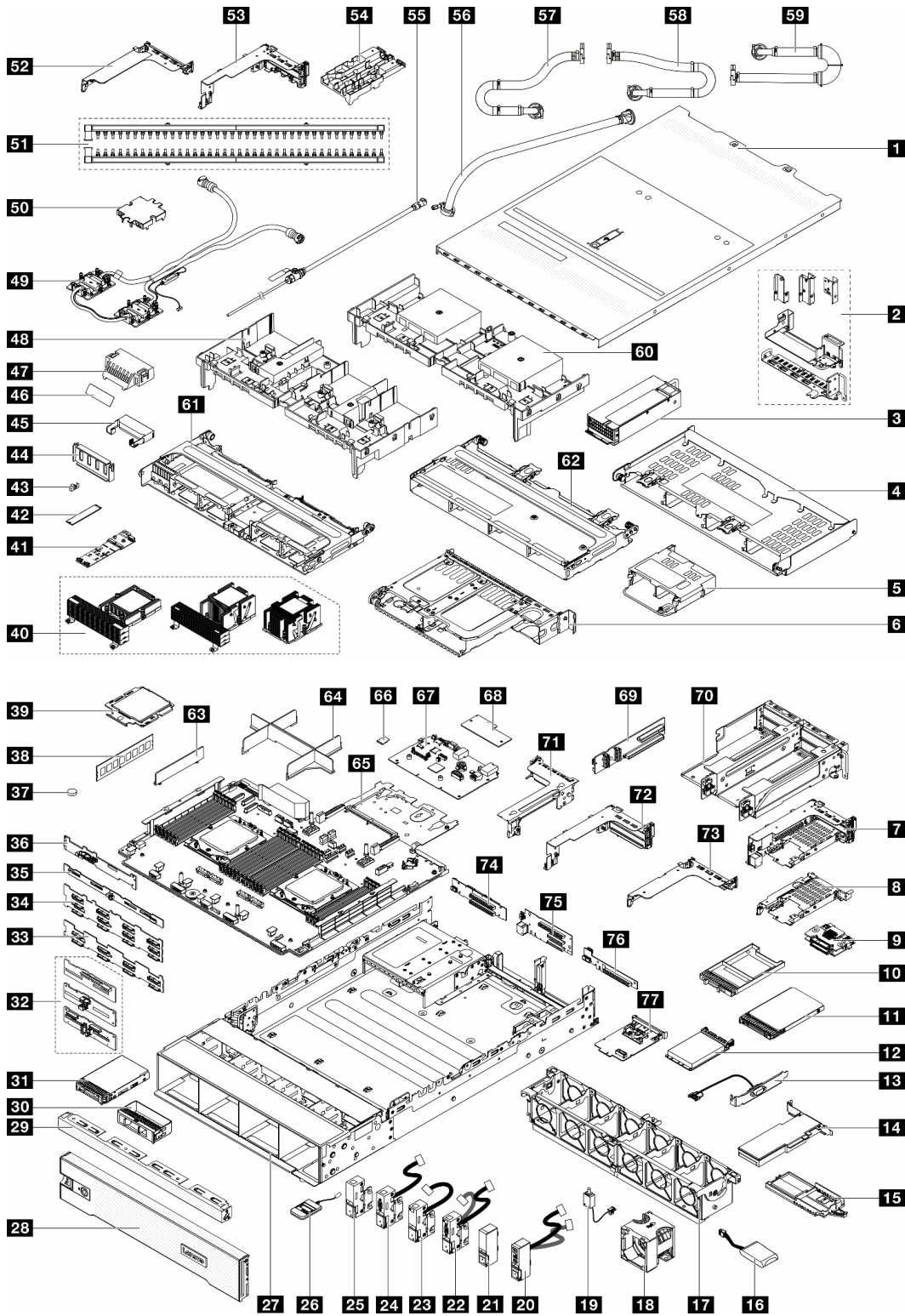
图 15. 服务器组件 (3.5 英寸硬盘插槽机箱)
