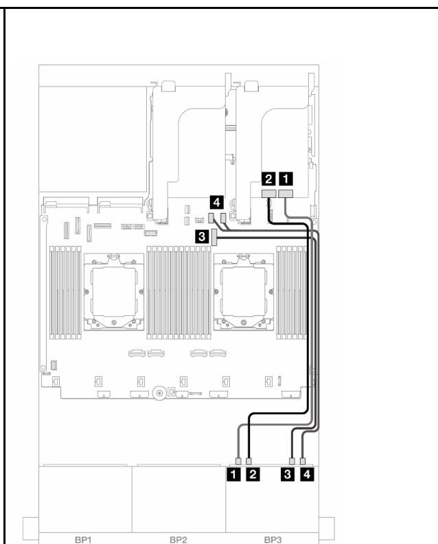
图 531. NVMe 线缆布放
