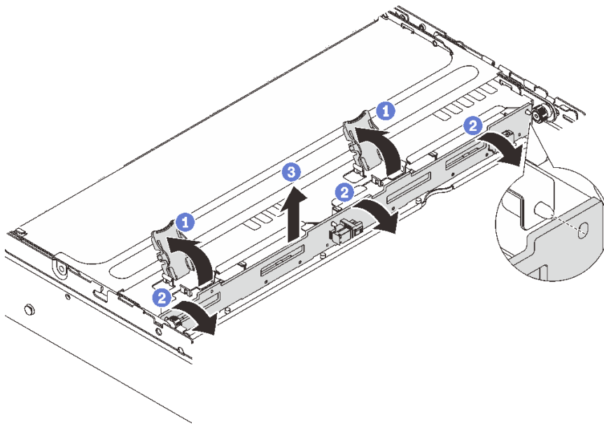
图 185. 卸下 3.5 英寸中间硬盘背板
