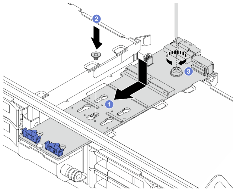
图 125. 将 M.2 背板安装到中间硬盘仓上
