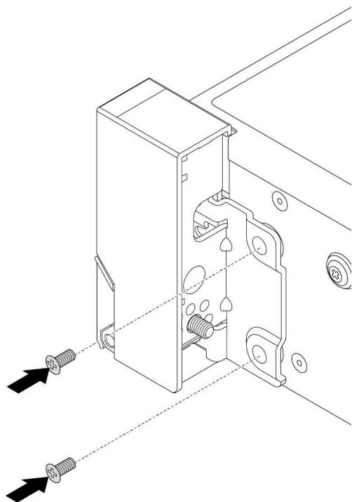
图 208. 安装螺钉
