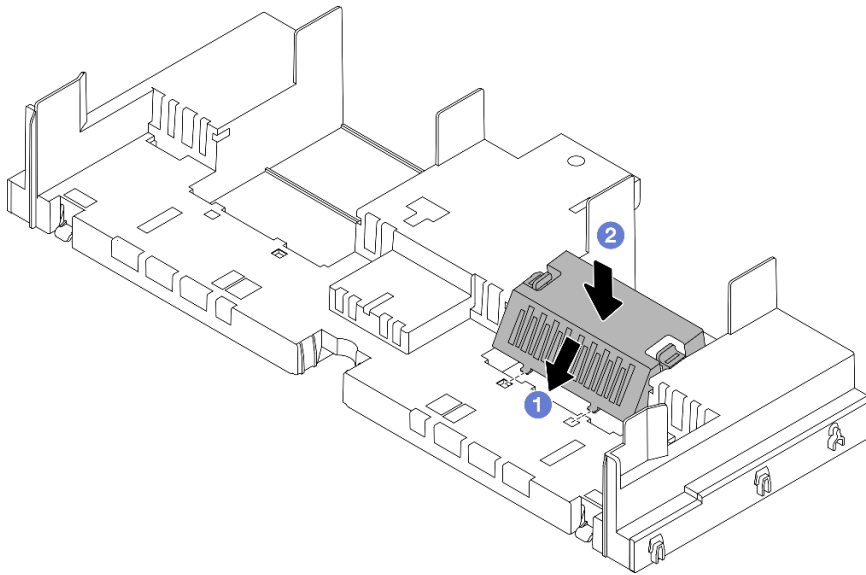
图 32. 安装导风罩填充件
