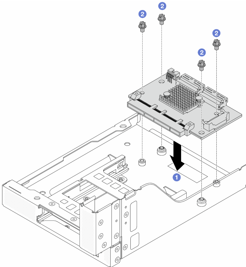
图 44. 安装正面 OCP 插转卡
