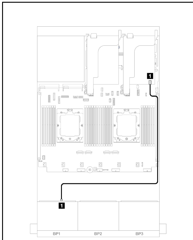
图 370. SAS/SATA 线缆布放
