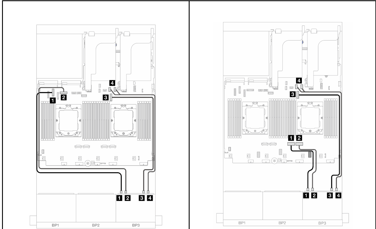
图 518. 装有两个处理器时的线缆布放
