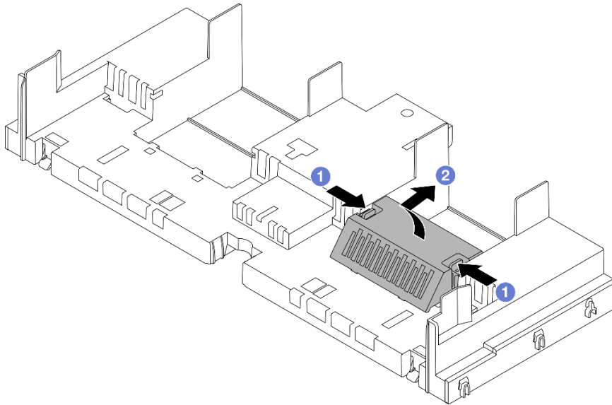
图 31. 卸下导风罩填充件
