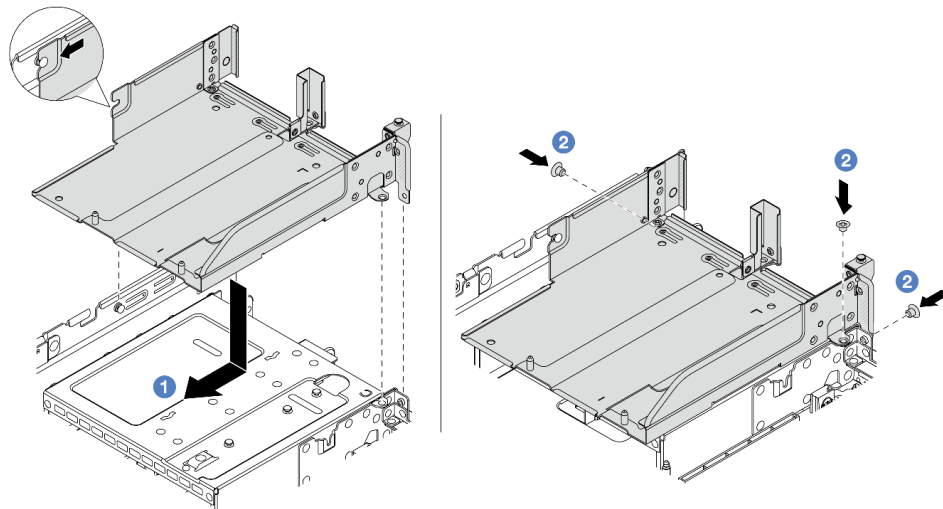
图 282. 安装转接卡架托盘
