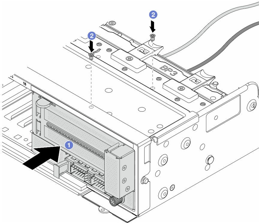
图 59. 安装正面适配器组合件
