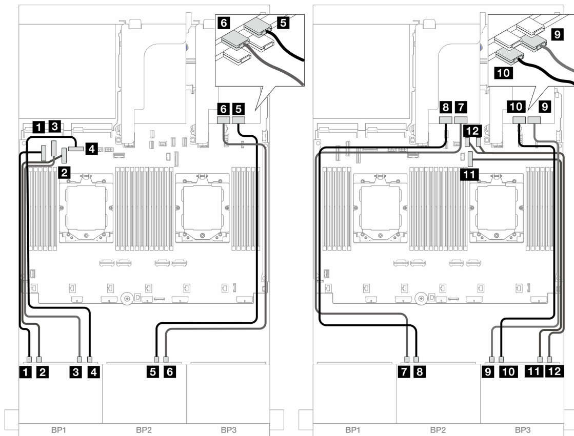
图 498. 到板载接口和重定时器卡的 NVMe 线缆布放
