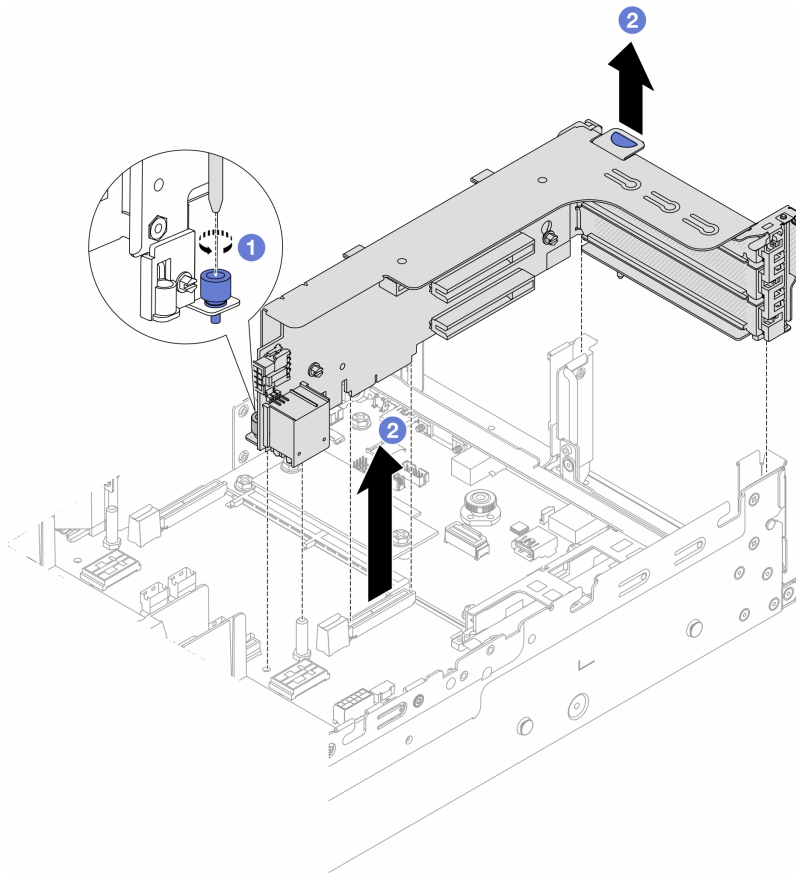
图 264. 卸下转接卡 1 组合件
