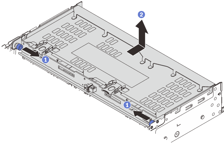
图 255. 卸下 4 x 3.5 英寸背面硬盘仓
