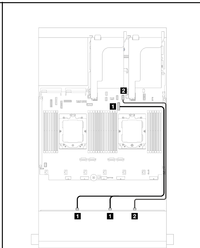
图 545. 装有一个处理器时到板载 SATA 接口的线缆布放
