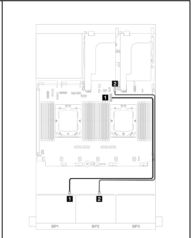
图 423. 装有一个处理器时的线缆布放
