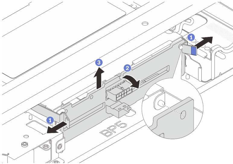
图 184. 卸下 2.5 英寸中间硬盘背板
