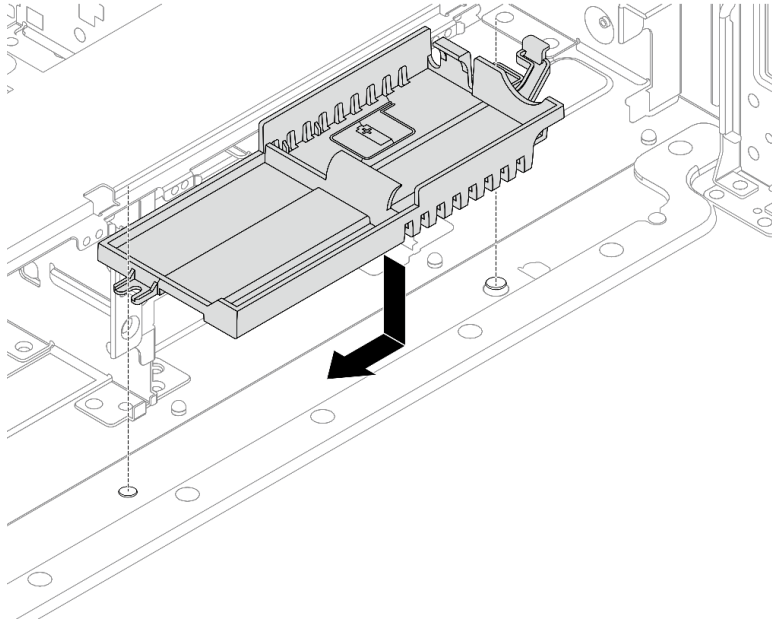
图 216. 安装超级电容器夹持器
