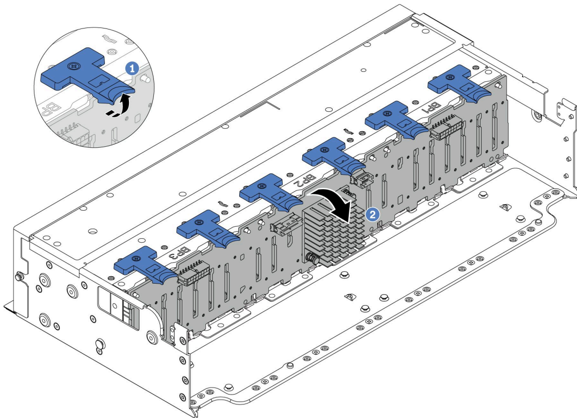
图 71. 卸下 24 插槽硬盘背板
