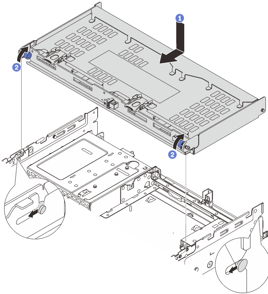
图 258. 安装 4 x 3.5 英寸背面硬盘仓
