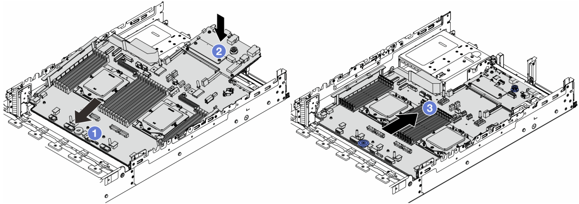
图 297. 安装主板组合件
