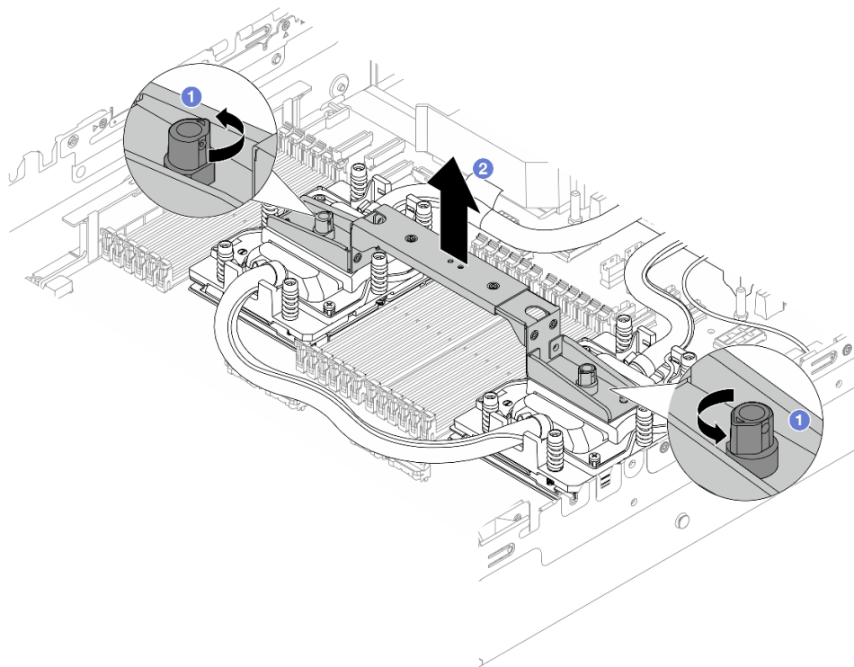
图 108. 卸下模块手柄
