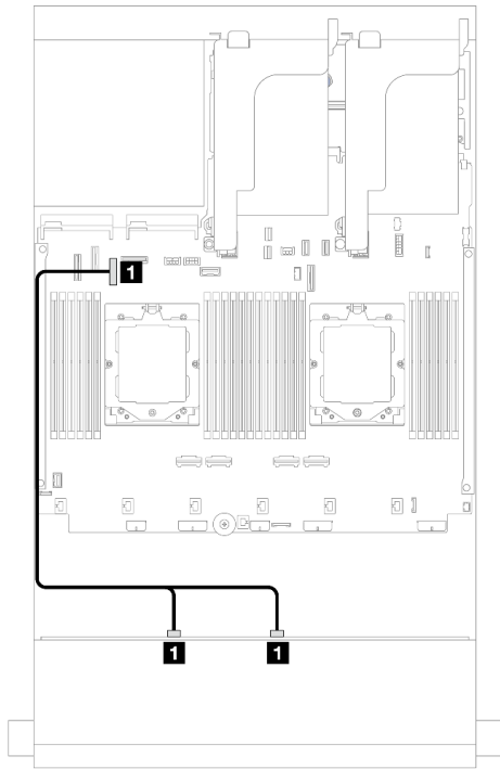
图 571. SAS/SATA 线缆布放
