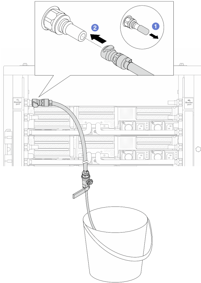
图 171. 将排气套件安装到供给侧
