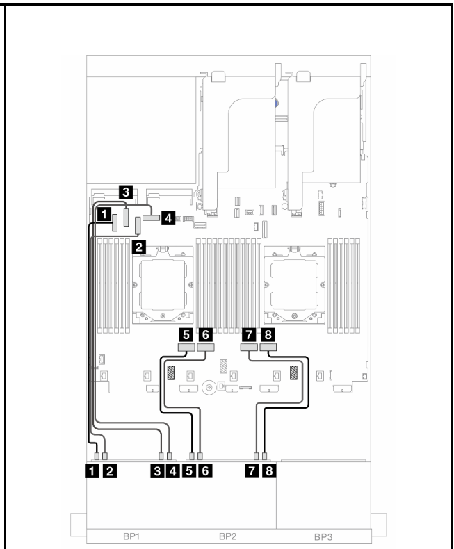
图 434. NVMe 线缆布放
