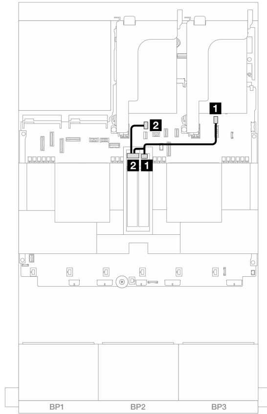
图 337. M.2 x1 RAID NVMe 2 插槽背板的线缆布放
