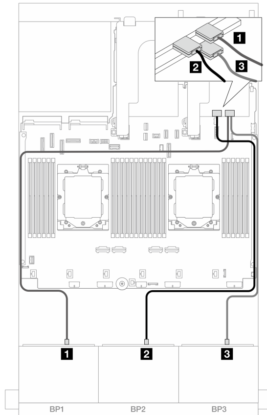
图 490. 到 8i/16i 三模式适配器的 SAS/SATA 线缆布放
