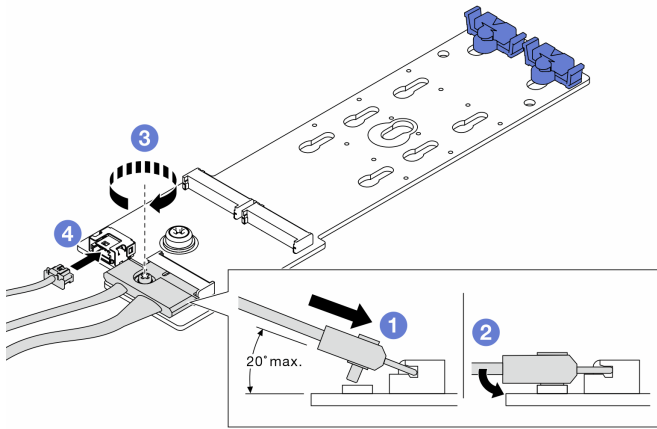
图 128. 将 M.2 线缆连接到 M.2 x1 RAID NVMe 2 插槽背板
