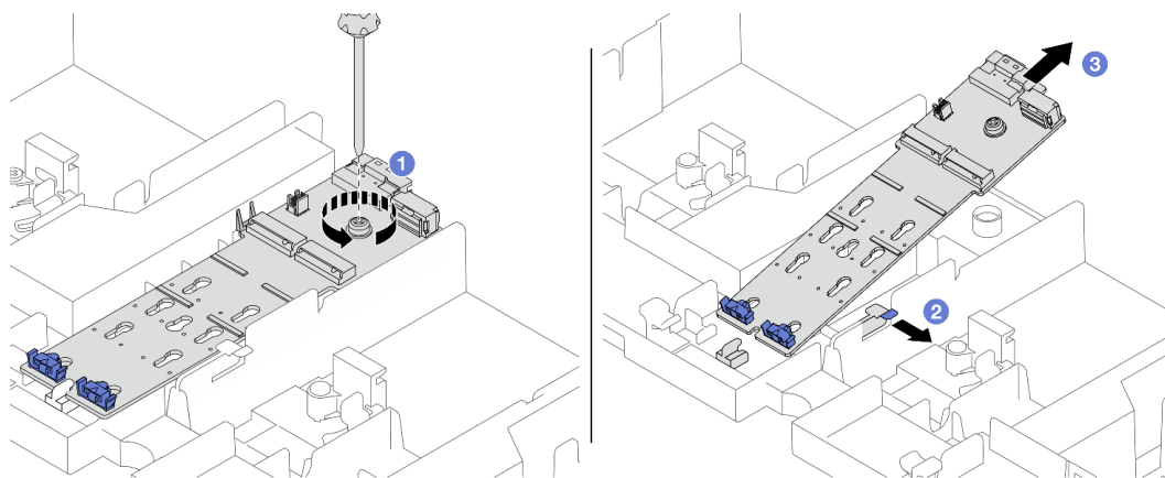
图 121. 从导风罩上卸下 M.2 背板
