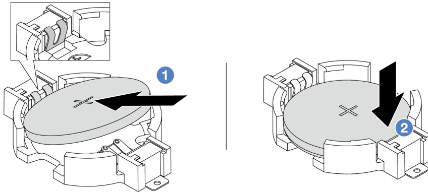
图 37. 安装 CMOS 电池
