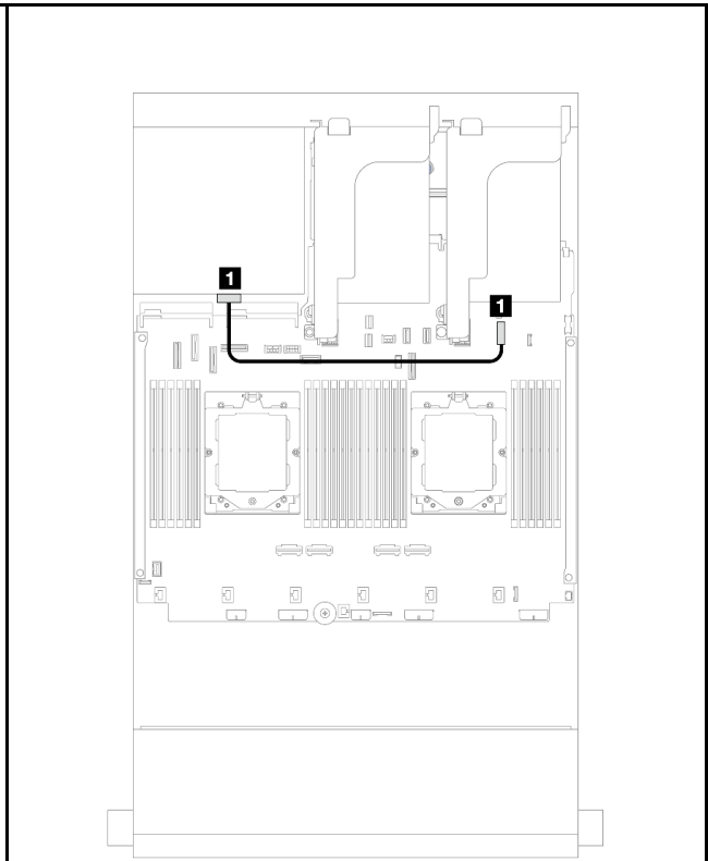
图 554. 背面背板电源线布放
