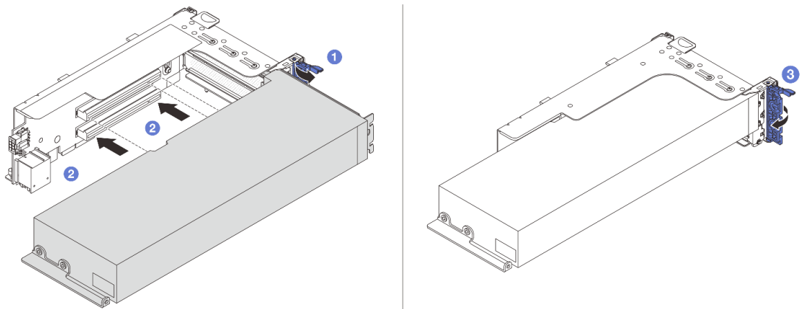
图 91. 安装 GPU 适配器
