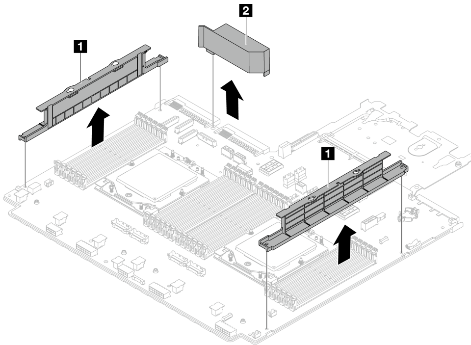
图 601. 从处理器板上卸下组件
