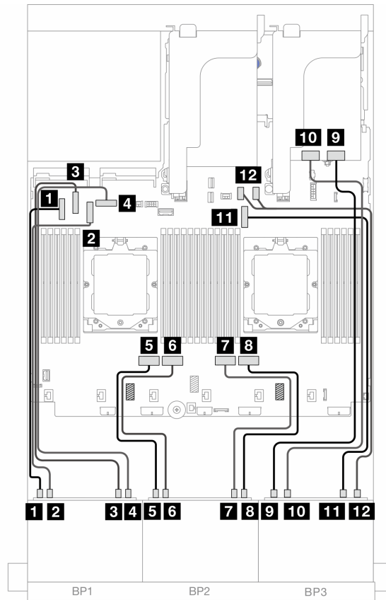
图 496. 到板载接口和重定时器卡的 NVMe 线缆布放
