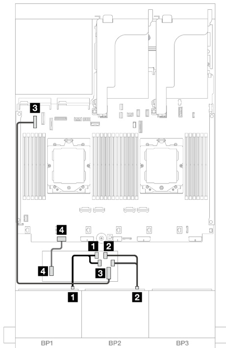
图 520. 到 CFF 适配器的线缆布放
