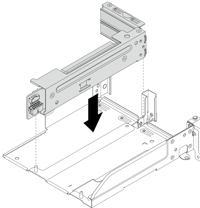
图 283. 安装转接卡 3/4 组合件
