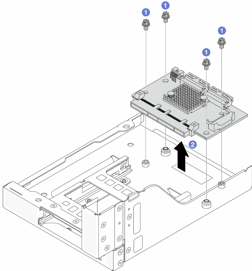
图 55. 卸下正面 OCP 插转卡
