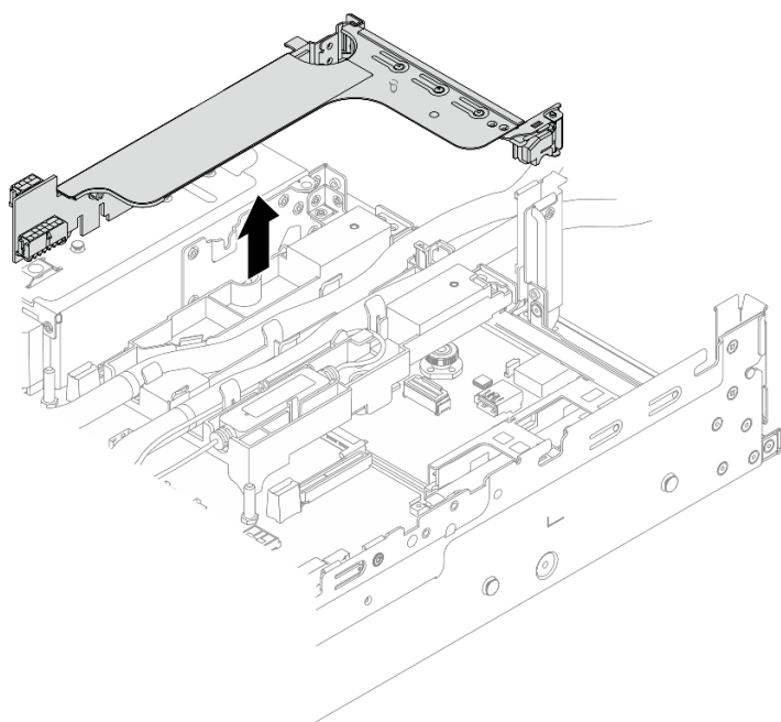
图 101. 卸下 1FH 转接卡架
