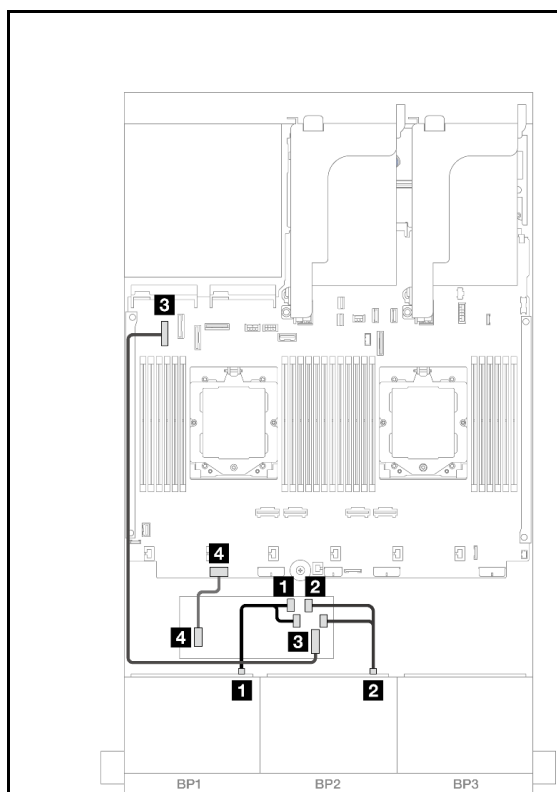
图 391. 装有两个处理器时的线缆布放
