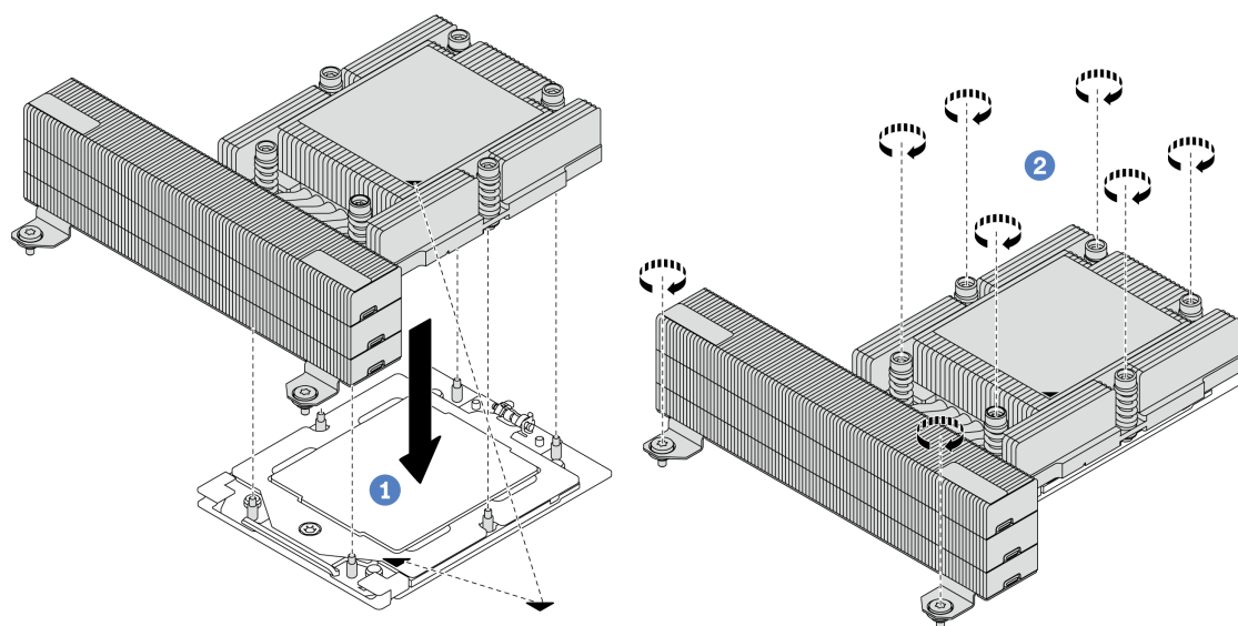
图 202. 安装高性能散热器
