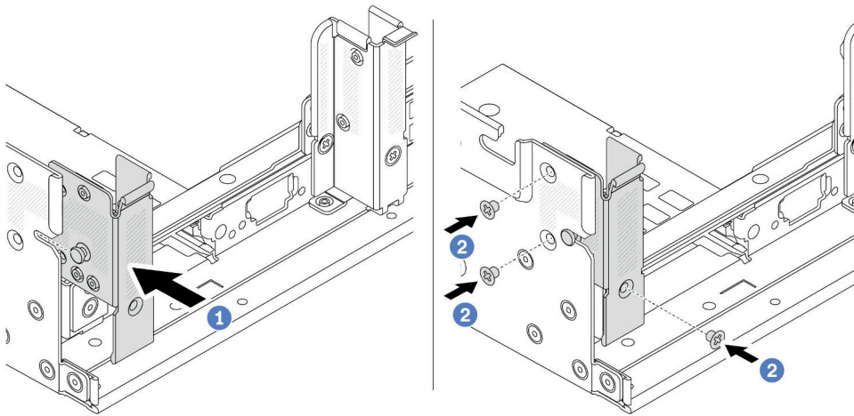
图 229. 安装 A1 背面壁挂支架（左侧）
