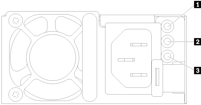
图 593. 电源模块 LED
