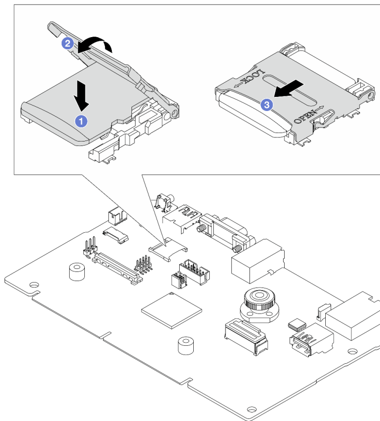
图 295. 安装 MicroSD 卡
