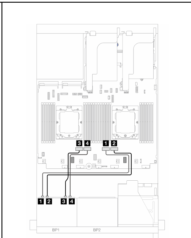
图 371. NVMe 线缆布放
