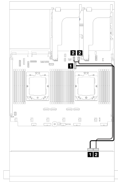
图 576. NVMe 线缆布放
