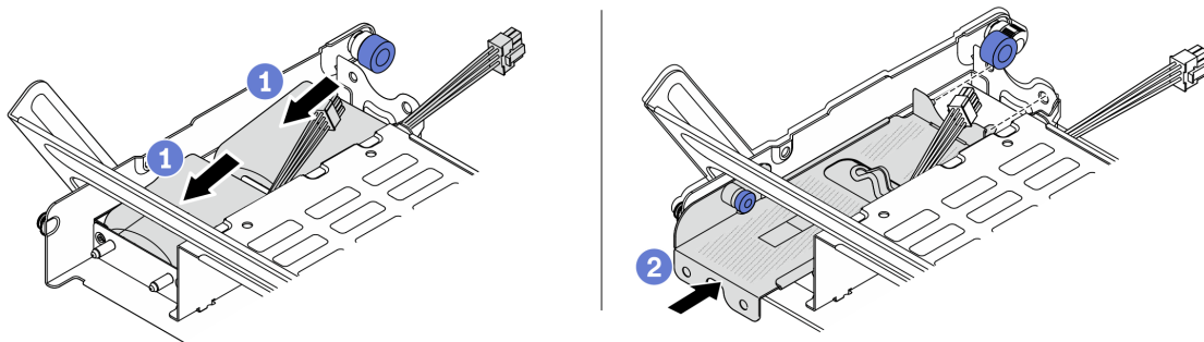
图 223. 将 RAID 快速充电模块安装到中间硬盘仓上
