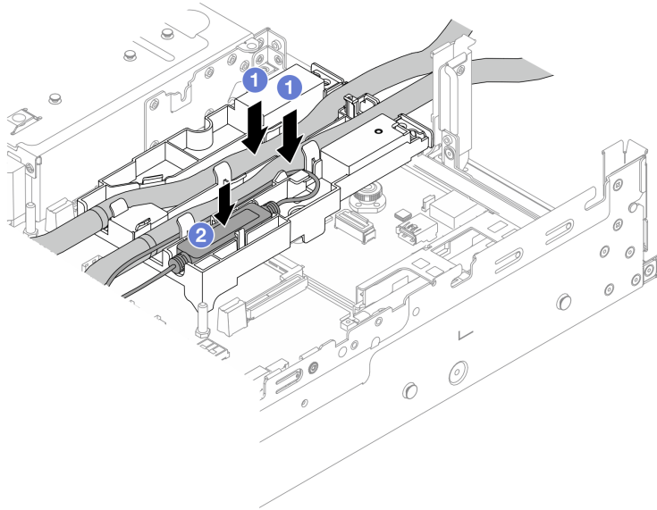
图 110. 放置软管和模块
