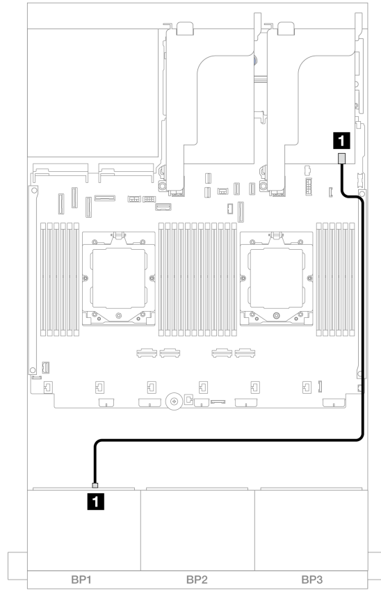
图 377. 到 8i RAID/HBA 适配器的 SAS/SATA 线缆布放
