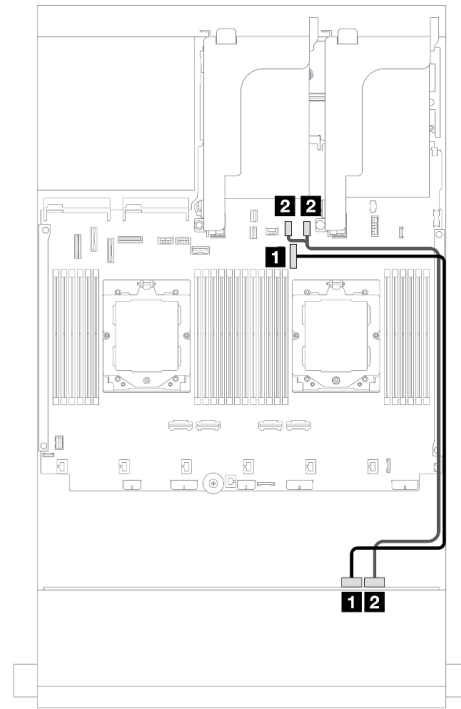
图 572. NVMe 线缆布放
