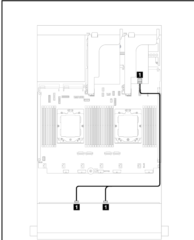
图 577. SAS/SATA 线缆布放
