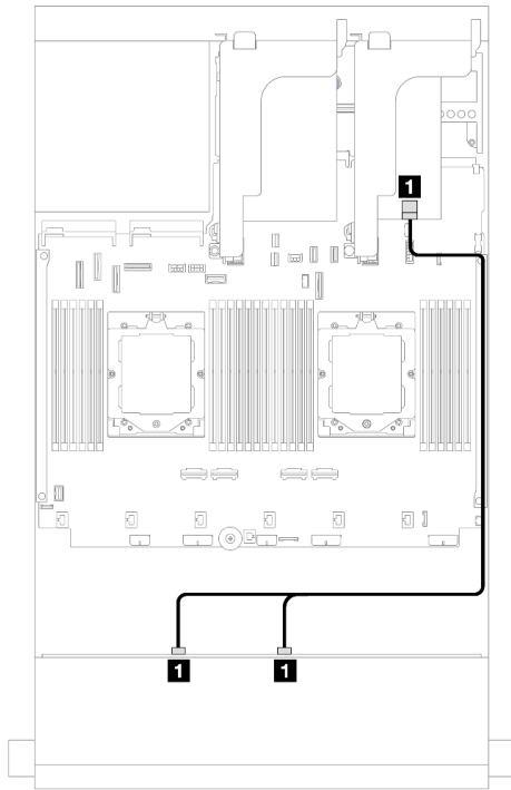
图 575. SAS/SATA 线缆布放
