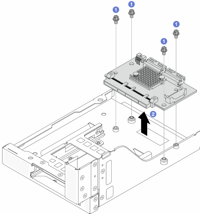
图 43. 卸下正面 OCP 插转卡
