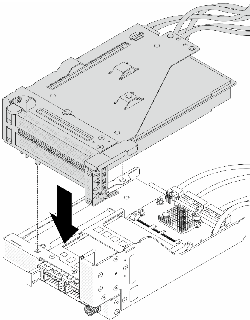
图 58. 将转接卡 5 组合件安装到正面 OCP 组合件上
