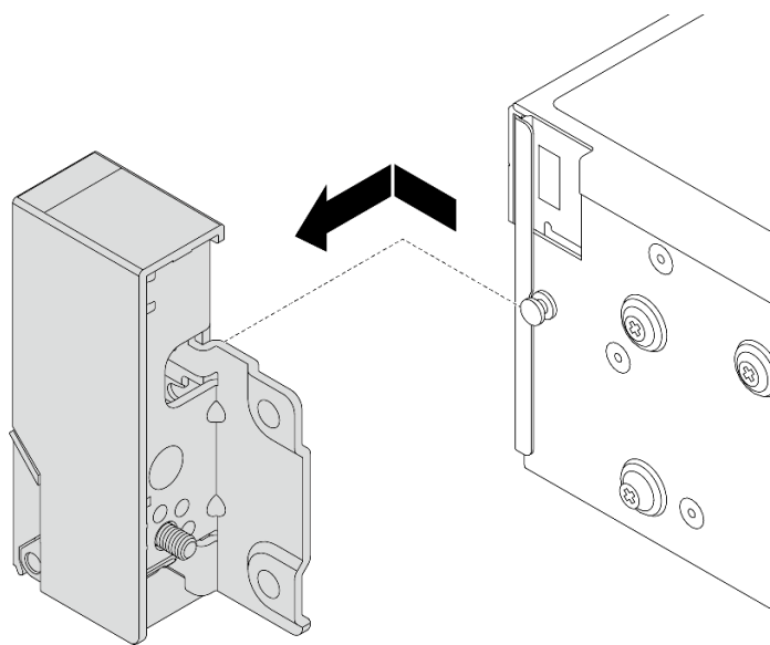
图 206. 卸下机架滑锁
