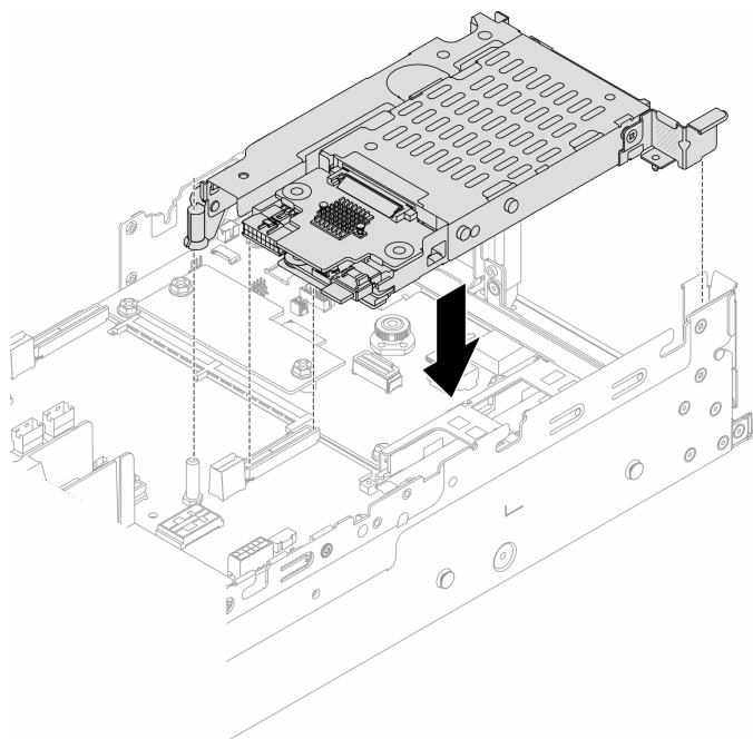
图 242. 安装 7 毫米固态硬盘转接卡架
