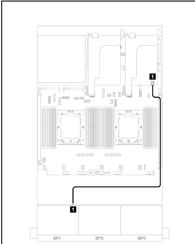
图 431. SAS/SATA 线缆布放
