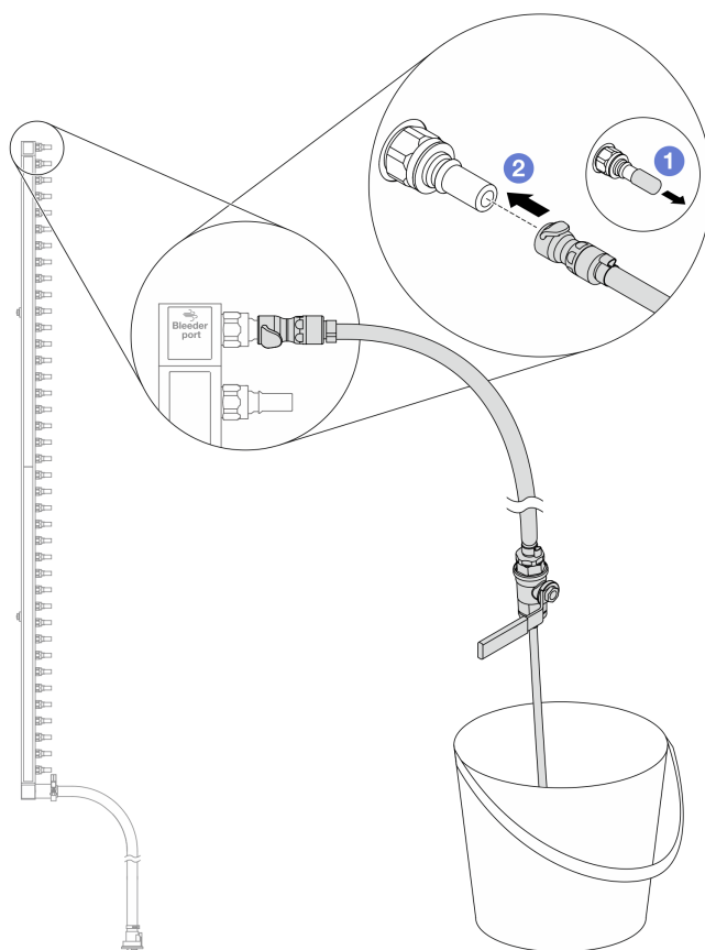
图 163. 将排气套件安装到供给侧
