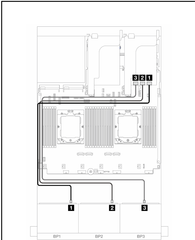
图 510. SAS/SATA 线缆布放
