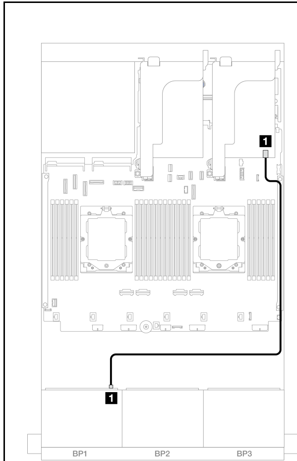
图 501. SAS/SATA 线缆布放
