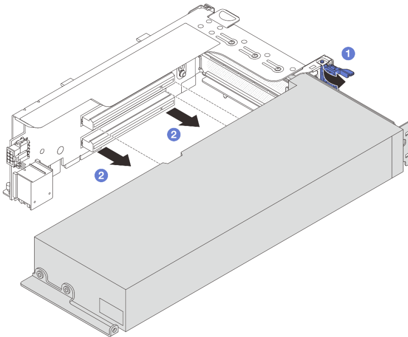
图 90. 卸下 GPU 适配器
