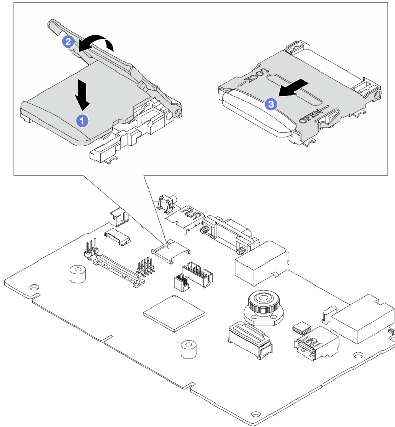
图 182. 安装 MicroSD 卡
