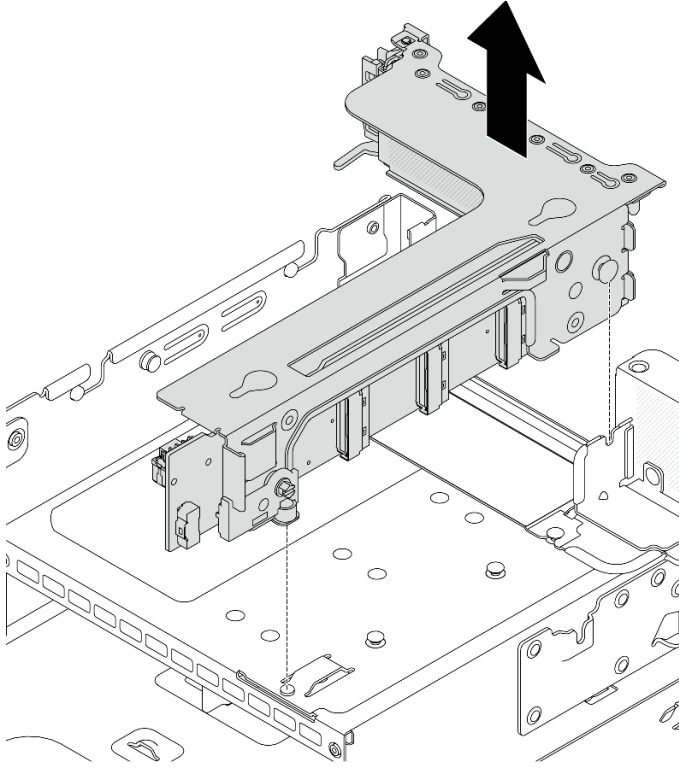
图 265. 卸下转接卡 3 组合件
