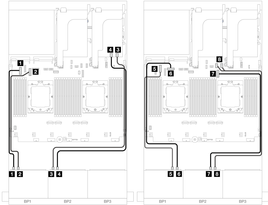
图 436. 到板载接口和重定时器卡的 NVMe 线缆布放
