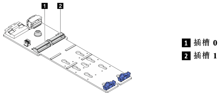
图 116. M.2 硬盘插槽
