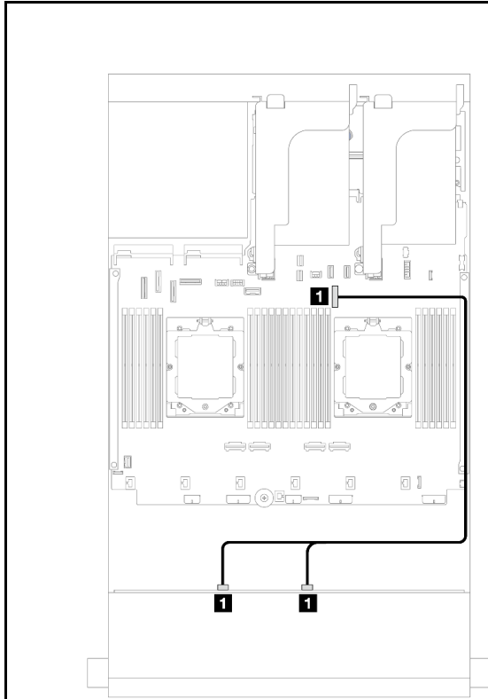
图 573. SAS/SATA 线缆布放
