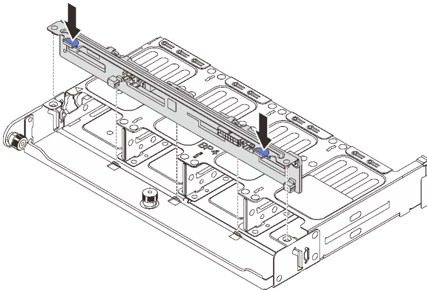
图 249. 安装 8 x 2.5 英寸背面硬盘背板
