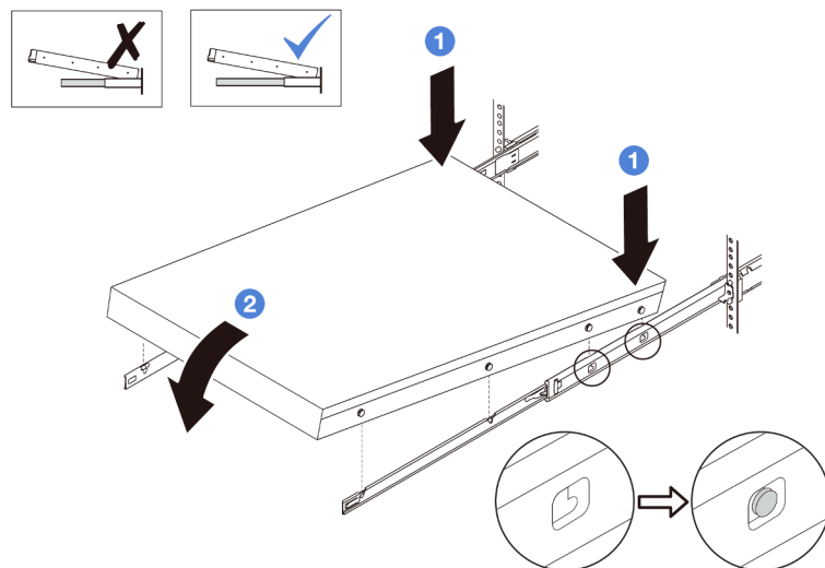
图 26. 将服务器装入导轨
