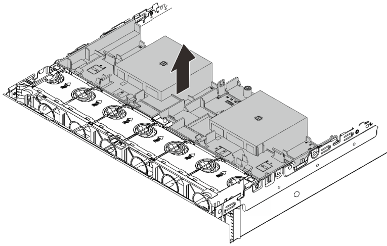
图 30. 卸下导风罩
