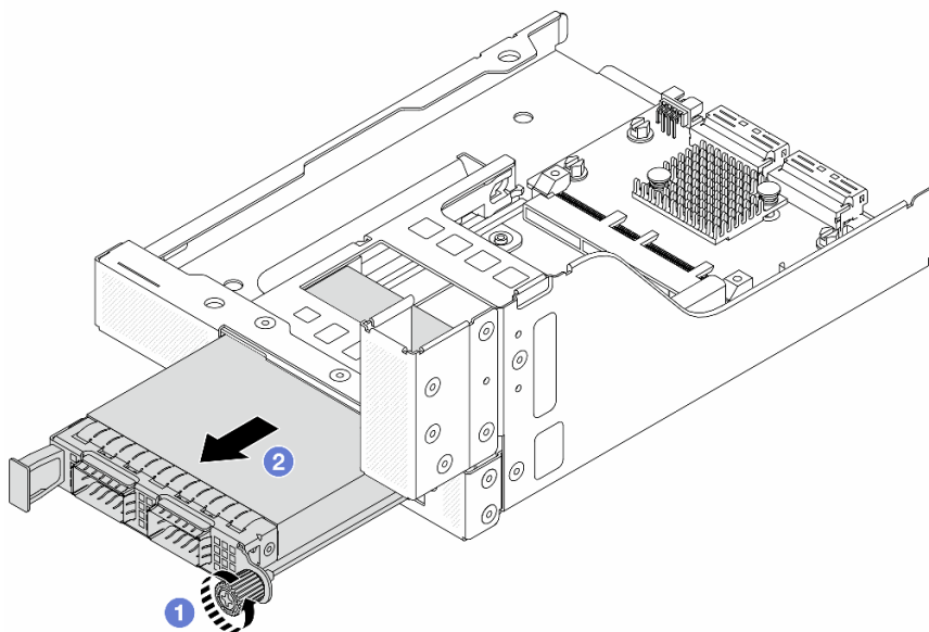
图 42. 卸下 OCP 模块
