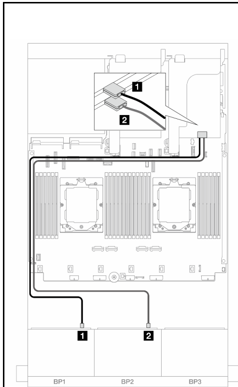
图 524. SAS/SATA 线缆布局
