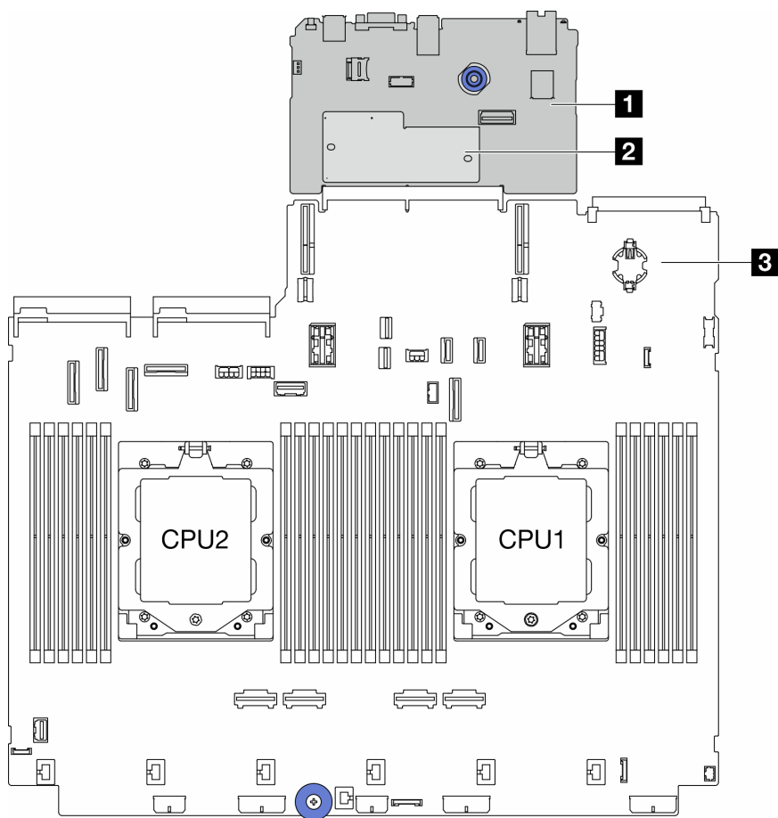
图 289. 主板组合件布局
