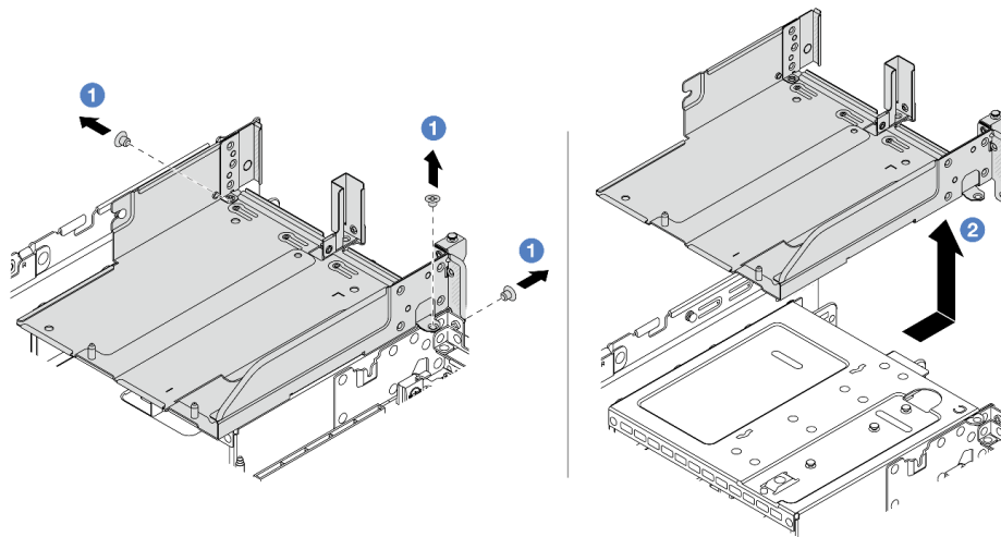
图 267. 卸下转接卡架托盘
