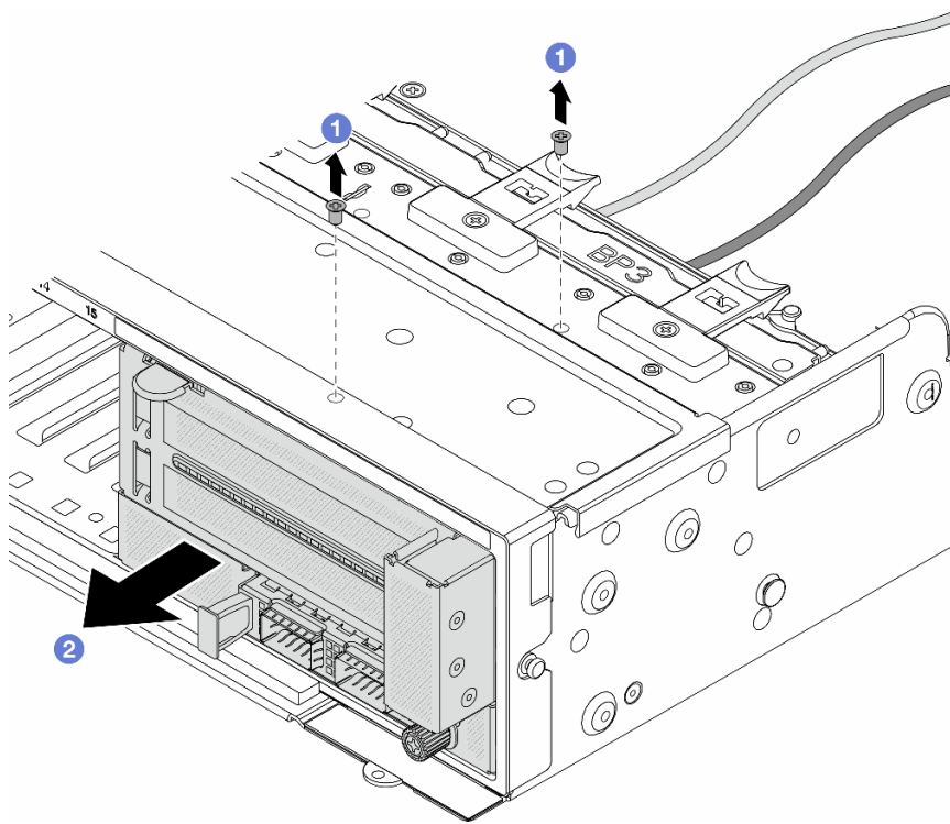
图 38. 卸下正面适配器组合件
