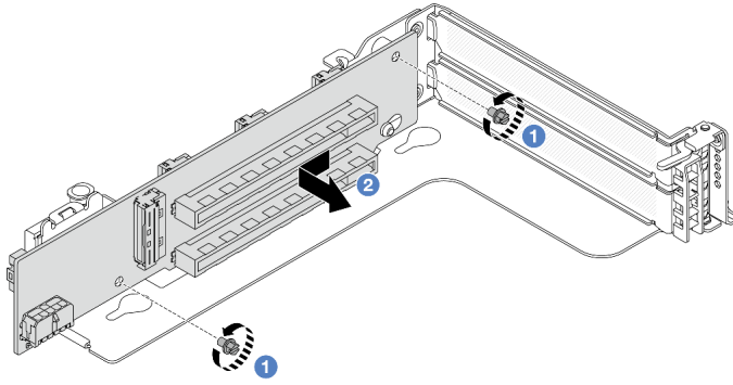
图 272. 从转接卡 3 架上卸下转接卡
