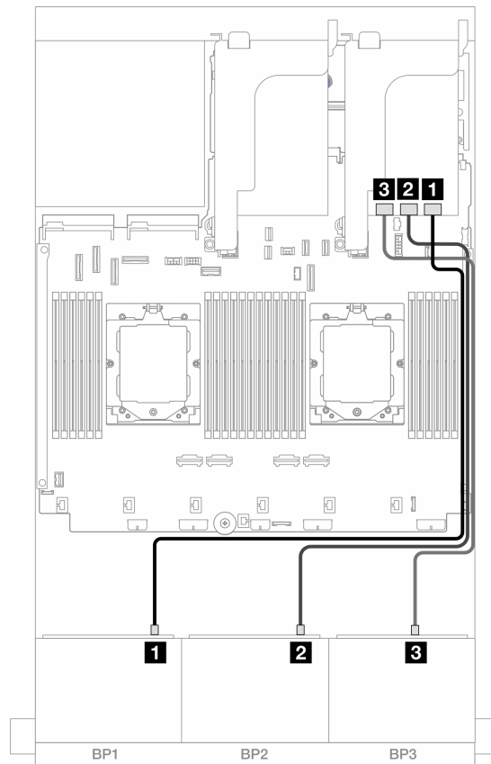
图 503. 到 32i 适配器的 SAS/SATA 线缆布放
