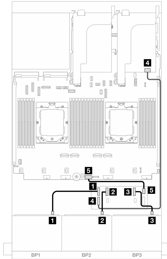
图 479. 到 CFF 扩展器和 8i/16i 适配器的 SAS/SATA 线缆布放
