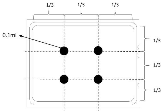
图 200. 涂抹导热油脂
