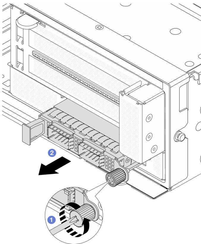
图 50. 卸下正面 OCP 模块
