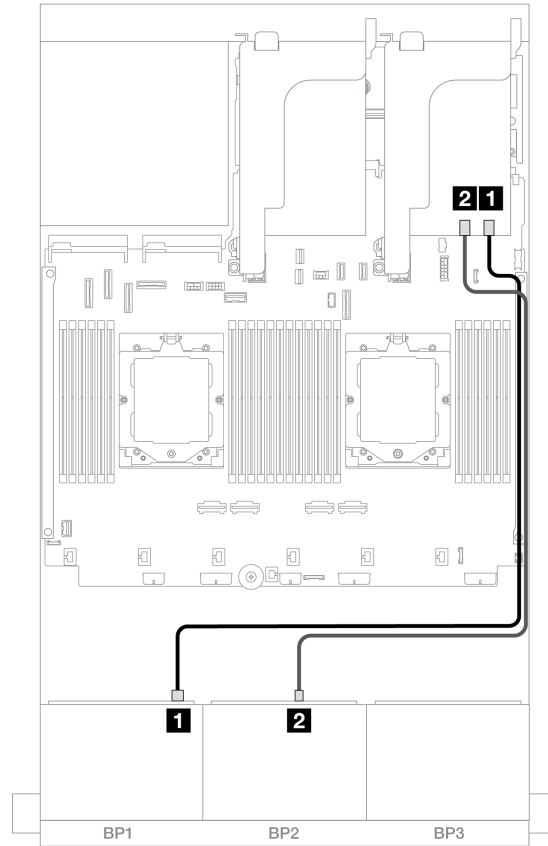
图 409. 到 16i 适配器的 SAS/SATA 线缆布放
