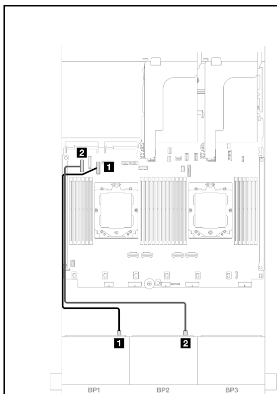
图 388. 装有两个处理器时的线缆布放
