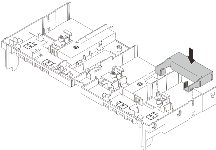
图 92. 安装附加导风罩 1
