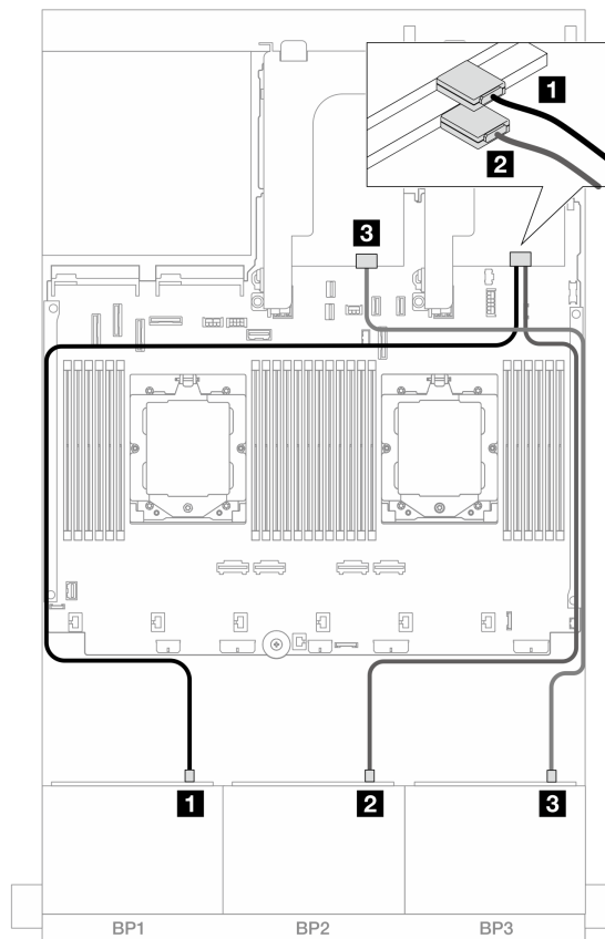
图 438. 到 8i 适配器的 SAS/SATA 线缆布放
