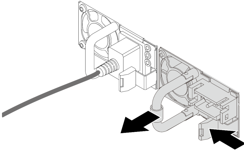
图 190. 卸下电源模块单元
