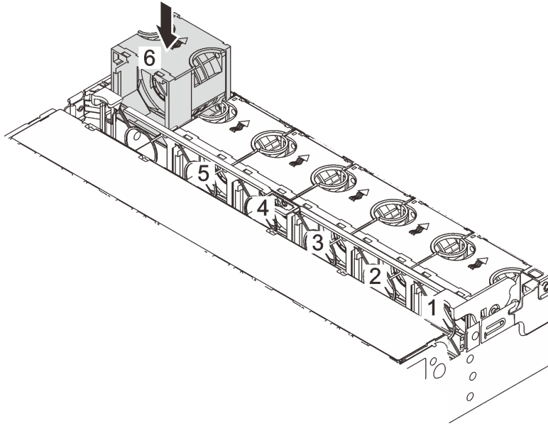
图 299. 安装系统风扇
