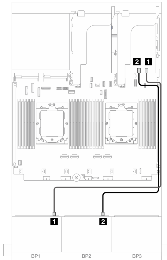
图 390. 到 16i RAID/HBA 适配器的 SAS/SATA 线缆布放
