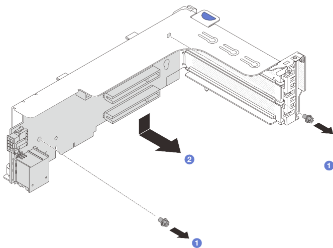
图 271. 从转接卡 1 架或转接卡 2 架上卸下转接卡
