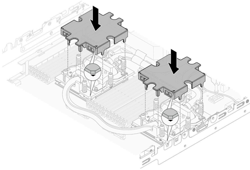
图 109. 安装冷却板外盖
