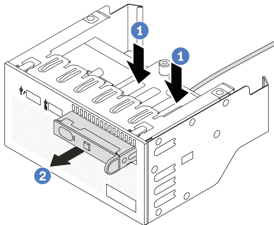
图 80. 卸下集成诊断面板
