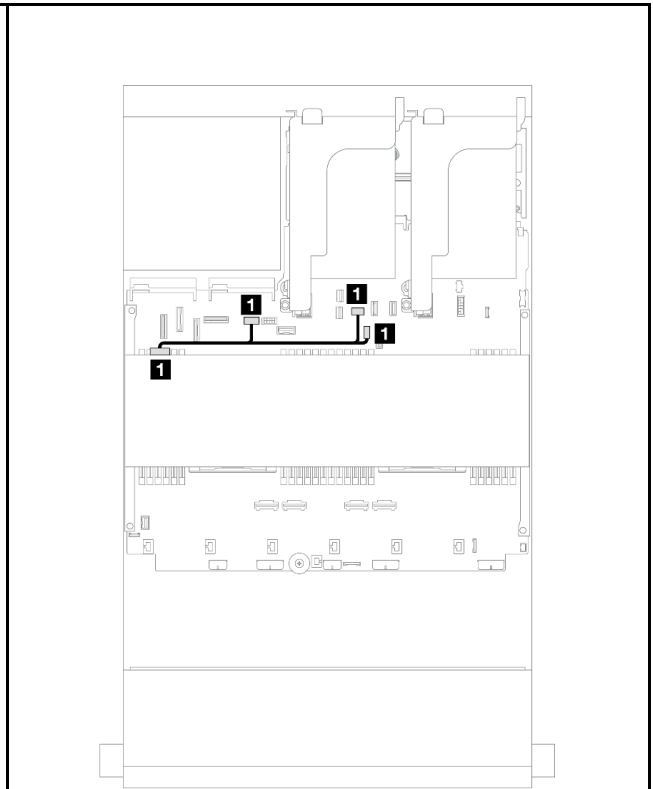
图 559. 中间背板电源线布放
