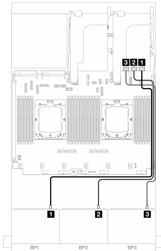
图 477. 到 32i 适配器的 SAS/SATA 线缆布放
