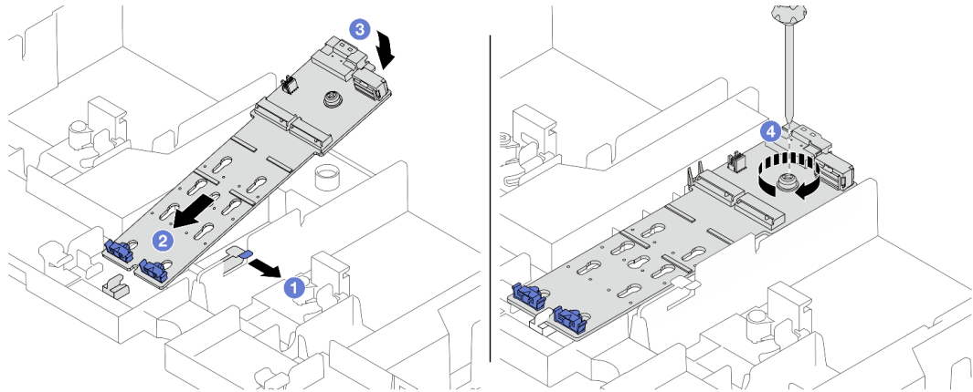
图 124. 将 M.2 背板安装到导风罩上
