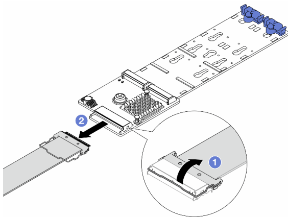
图 120. 从 M.2 RAID SATA/NVMe 2 插槽背板上拔下线缆
