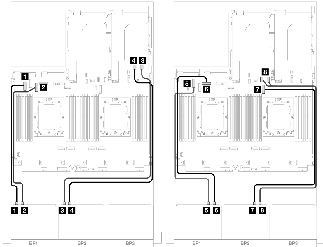
图 405. 到板载接口和重定时器卡的 NVMe 线缆布放
