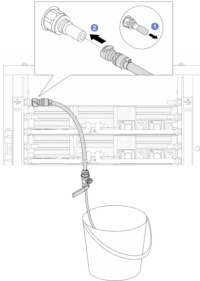
图 154. 将排气套件安装到供给侧
