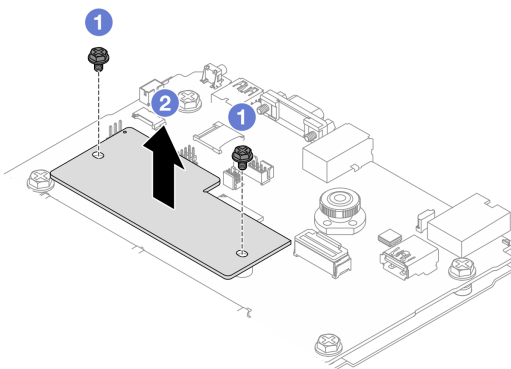
图 290. 卸下固件和 RoT 安全模块
