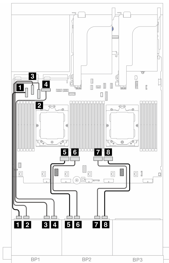
图 404. 到板载 PCIe 接口的 NVMe 线缆布放
