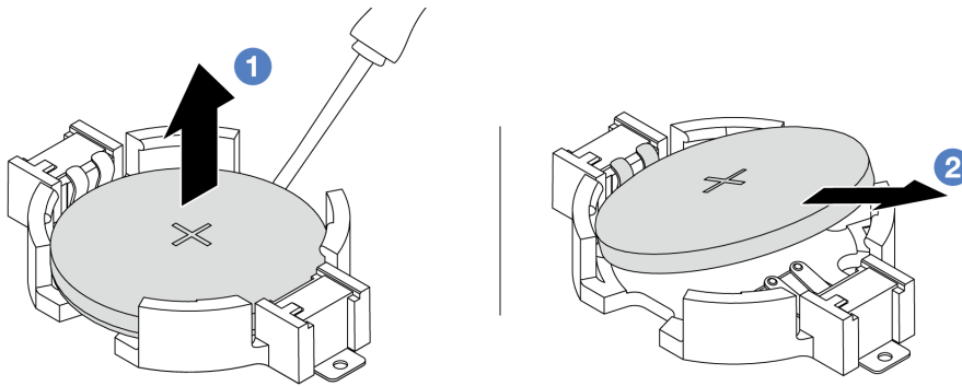
图 36. 卸下 CMOS 电池
