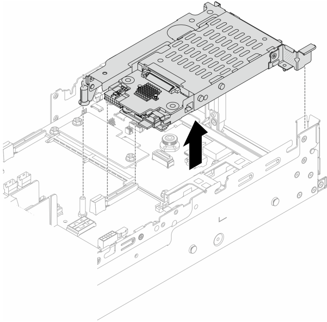
图 233. 卸下 7 毫米固态硬盘转接卡架
