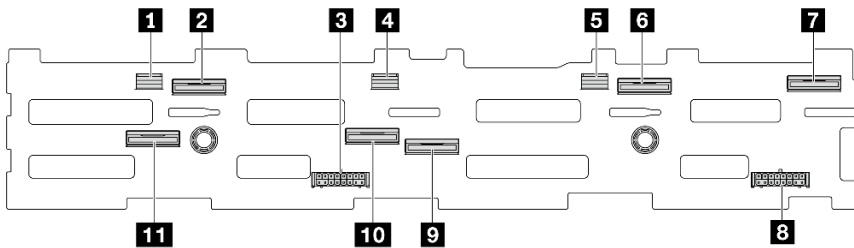
图 317. 12 x 3.5 英寸 AnyBay 背板接口
