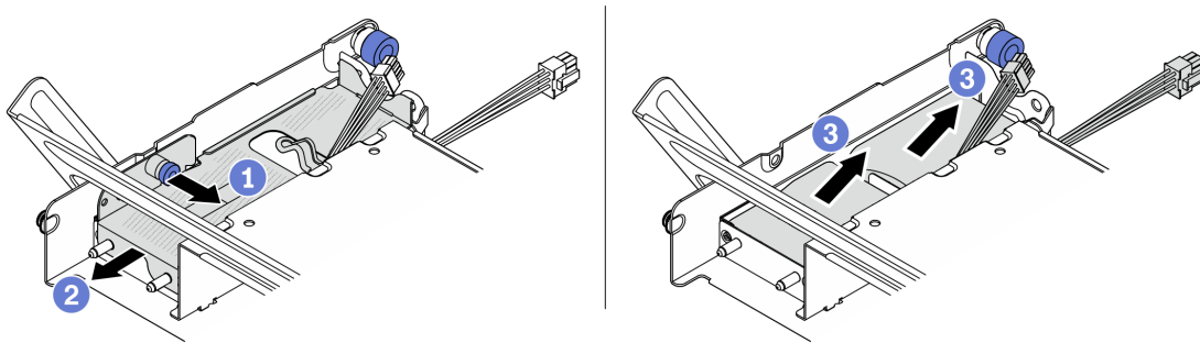
图 222. 从中间硬盘仓上卸下 RAID 快速充电模块
