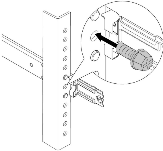
图 28. 将服务器固定到机架背面
