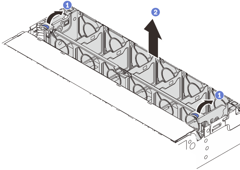
图 300. 卸下系统风扇架
