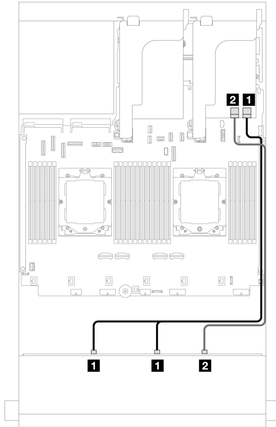
图 546. 到一个 16i RAID/HBA 适配器的线缆布放
