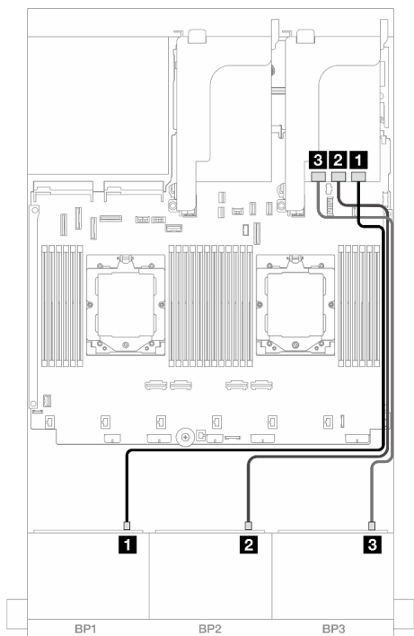
图 440. 正面背板线缆布放
