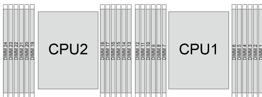
图 19. 内存条和处理器布局
