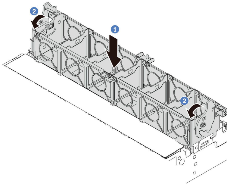
图 301. 安装系统风扇架
