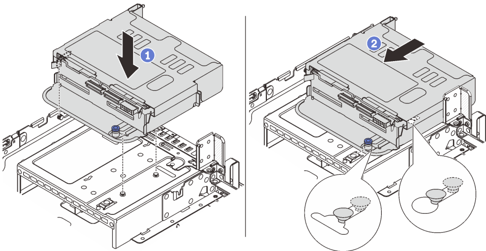
图 246. 安装 4 x 2.5 英寸背面硬盘仓
