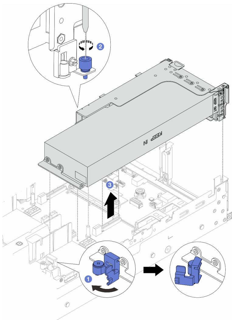
图 88. 卸下带有 GPU 适配器的转接卡 1 组合件
