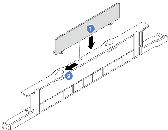
图 35. 安装 2U 线缆壁挂支架
