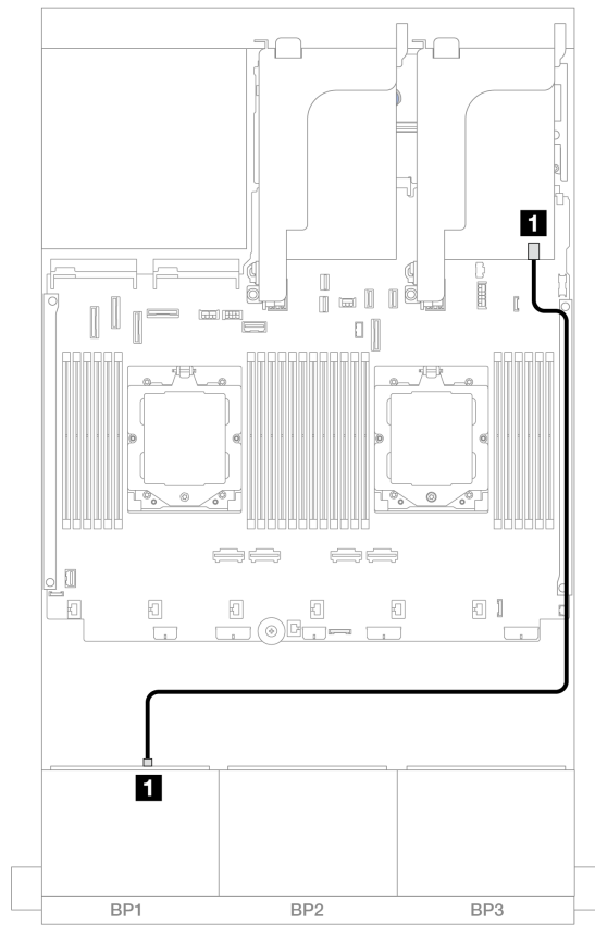
图 495. 到 8i 适配器的 SAS/SATA 线缆布放
