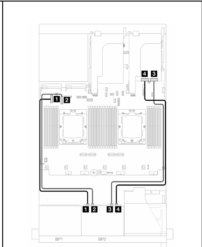
图 432. NVMe 线缆布放
