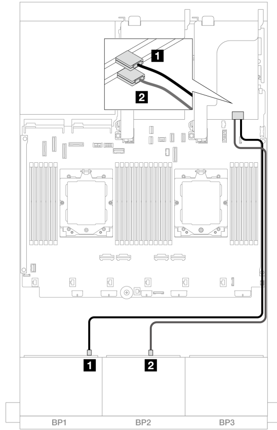
图 406. 到 8i 适配器的 SAS/SATA 线缆布放
