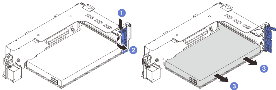
图 268. 从转接卡 1 或 2 组合件上卸下 PCIe 适配器
