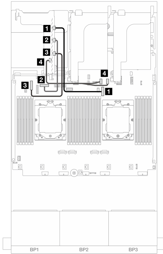
图 349. x16/x16 Gen 4 PCIe 转接卡 3 的信号线缆连接
