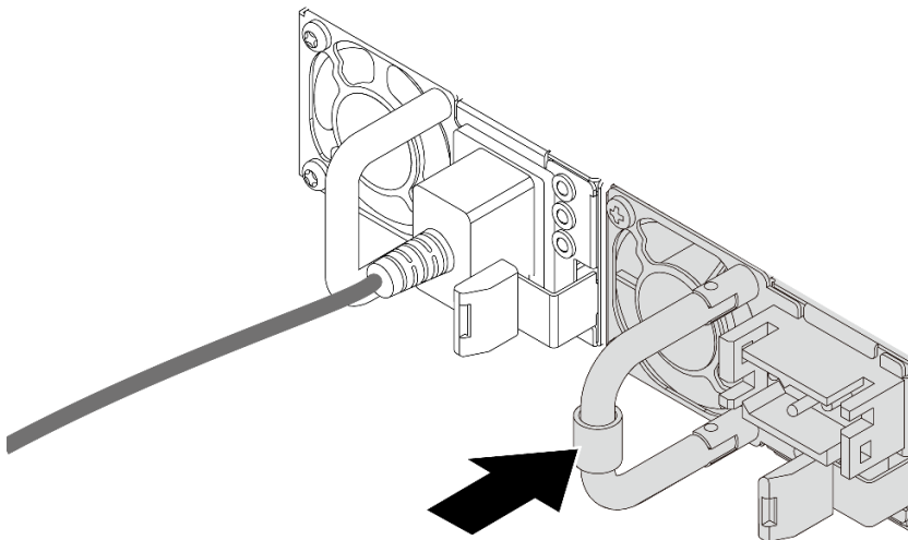
图 192. 安装电源模块单元
