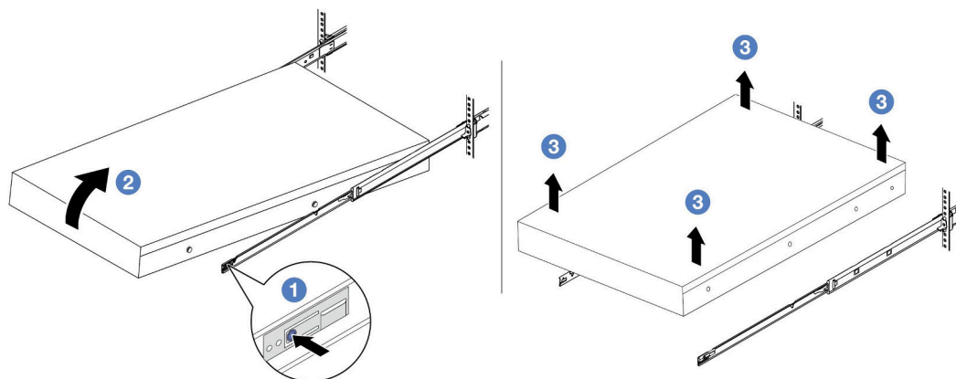
图 23. 从机架上卸下服务器
