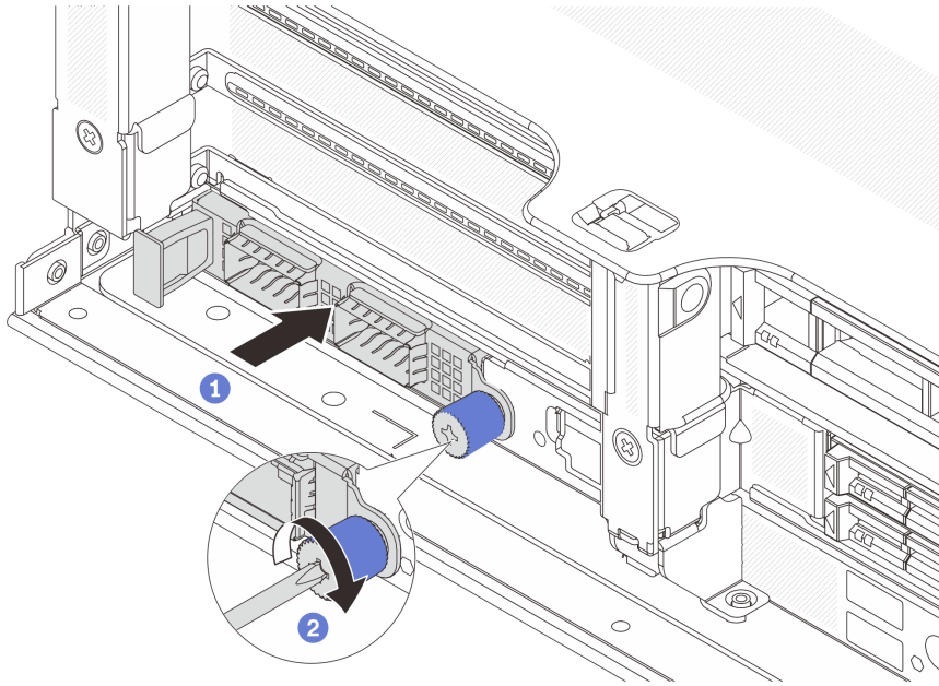
图 261. 安装背面 OCP 模块
