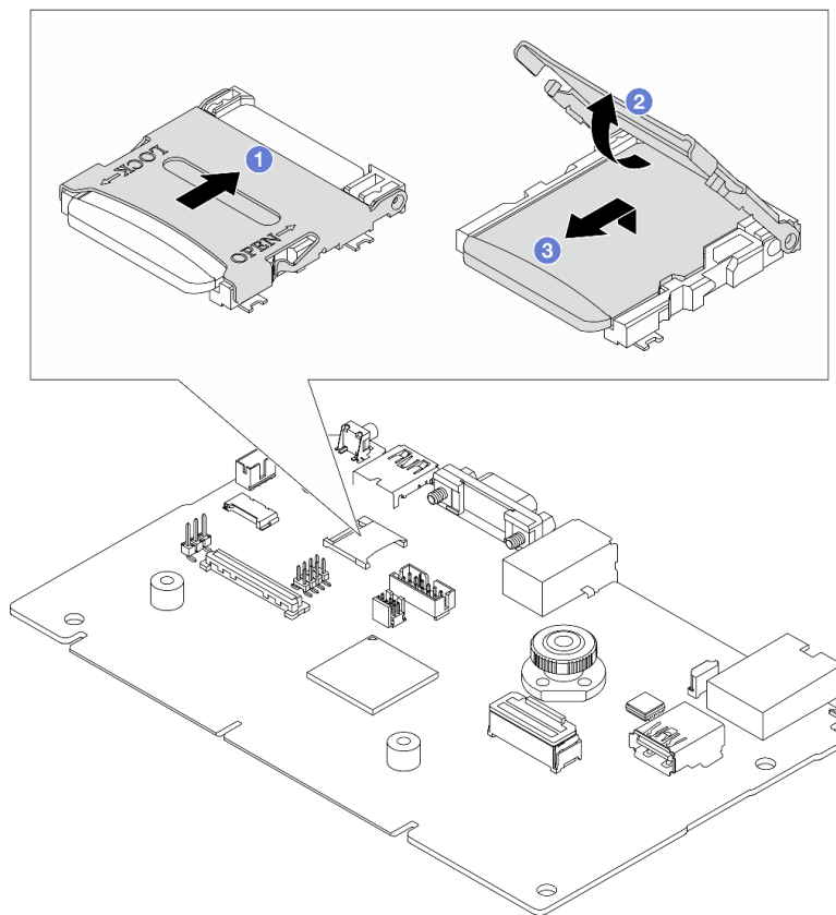
图 294. 卸下 MicroSD 卡
