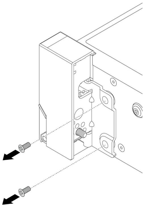
图 205. 卸下螺钉
