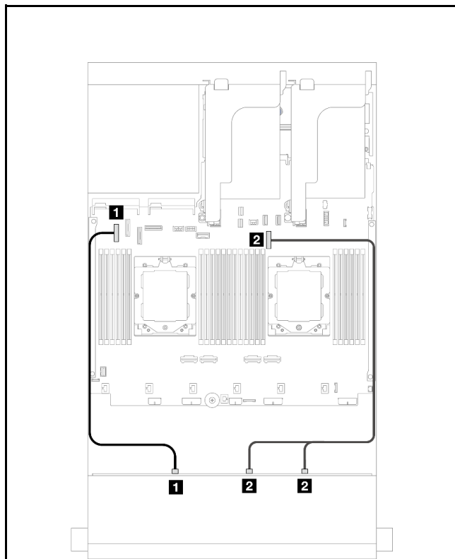
图 544. 装有两个处理器时到板载 SATA 接口的线缆布放
