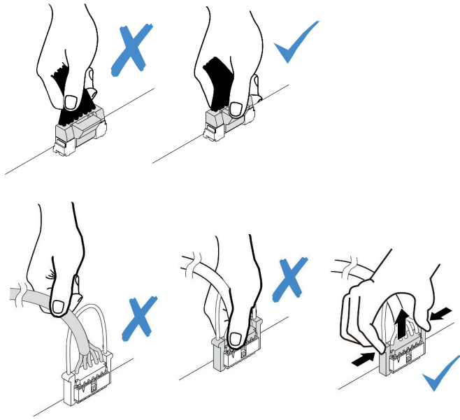
图 95. 从主板组合件上拔下线缆
