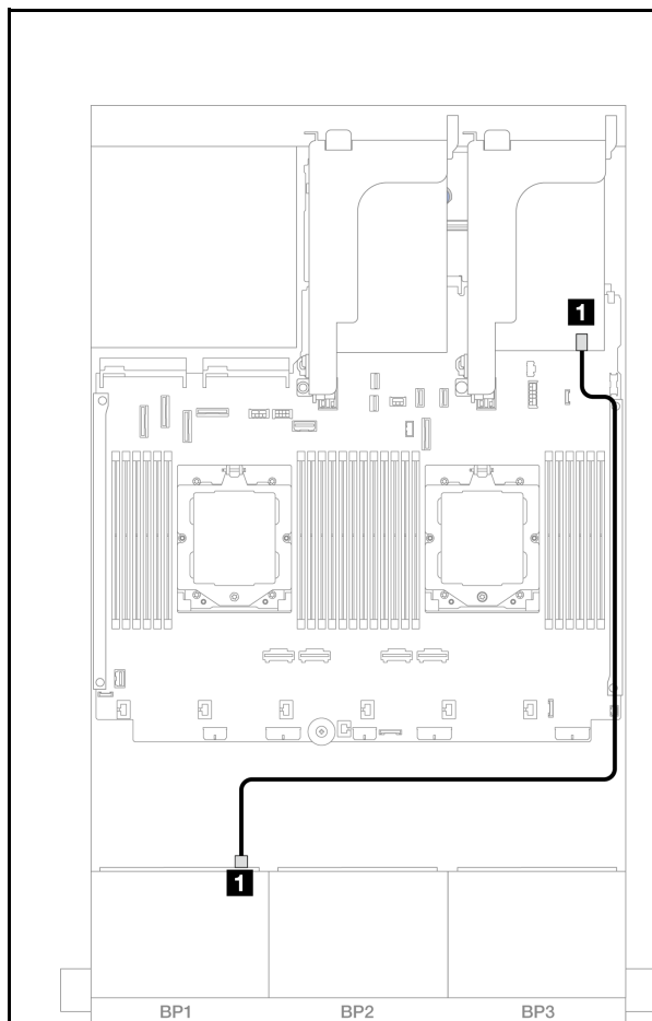
图 499. SAS/SATA 线缆布放
