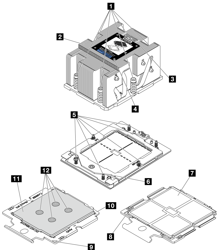
图 193. 处理器和散热器组件
