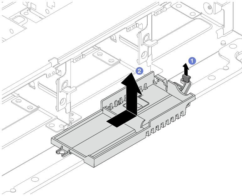
图 215. 卸下超级电容器夹持器
