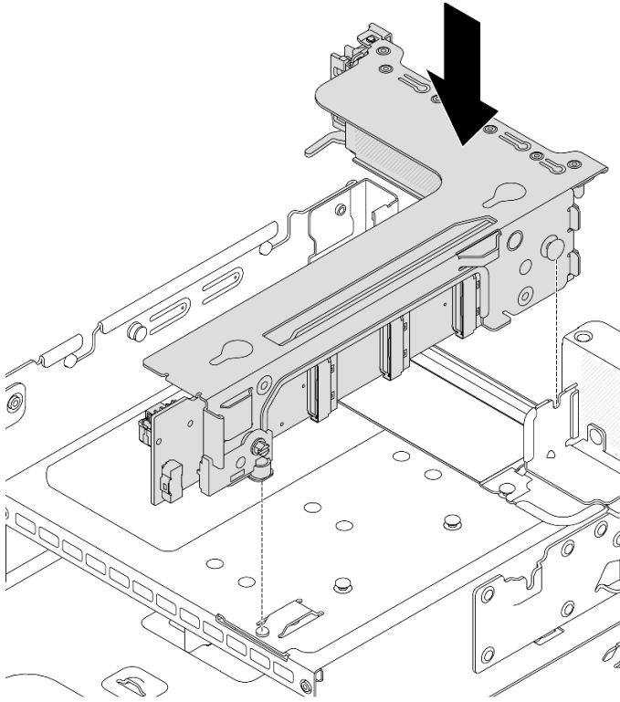
图 281. 安装转接卡 3 组合件
