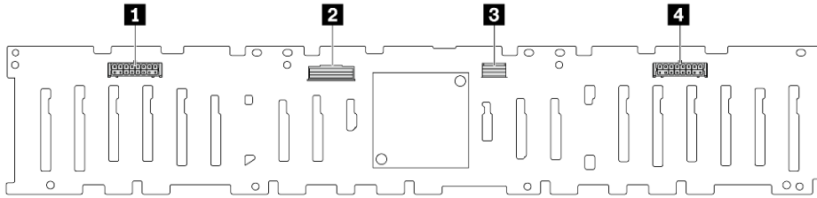
图 313. 24 x 2.5 英寸 SAS/SATA 扩展器背板上的接口
