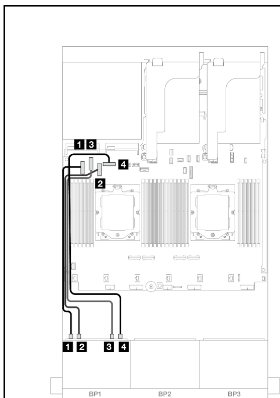
图 384. 装有两个处理器时的线缆布放
