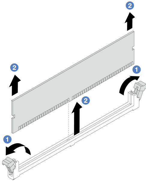
图 179. 卸下内存条
