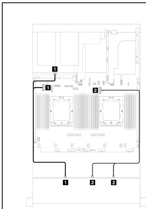
图 547. 装有两个处理器时的线缆布放
