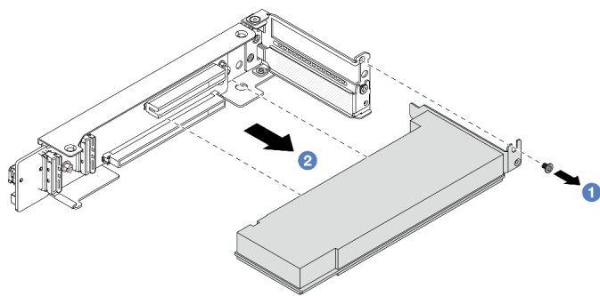
图 270. 从 4LP 转接卡 3/4 组合件上卸下 PCIe 适配器
