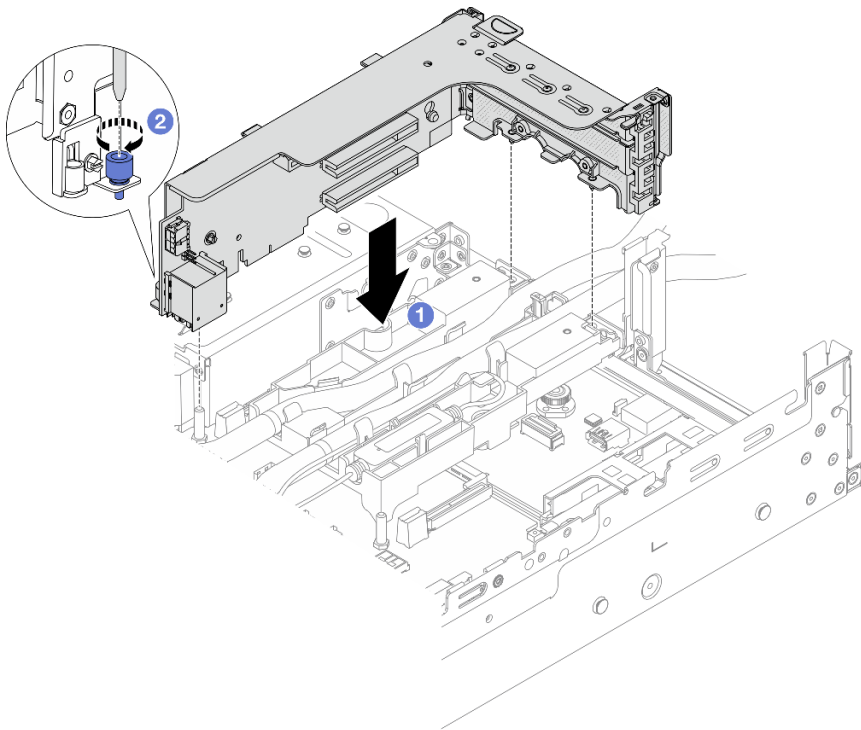
图 113. 安装 3FH 转接卡架
