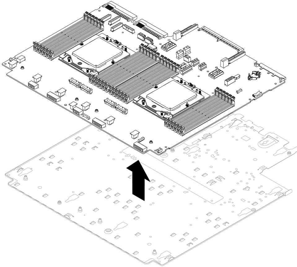
图 602. 将处理器板与支撑金属板分开
