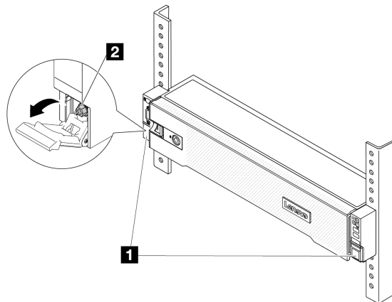
图 29. 将服务器固定到机架正面
