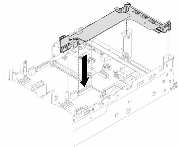
图 308. 安装转接卡组合件
