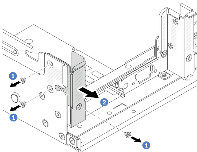
图 226. 卸下 A1 背面壁挂支架（左侧）
