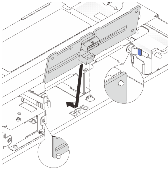
图 186. 安装 2.5 英寸中间硬盘背板
