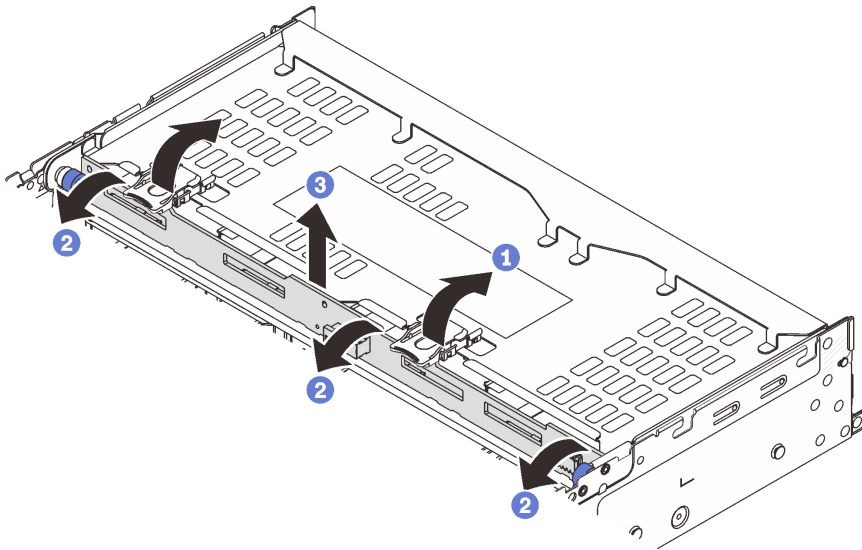
图 256. 卸下 4 x 3.5 英寸背面硬盘背板
