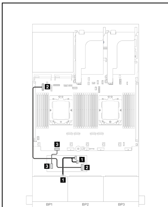
图 363. 装有两个处理器时的线缆布放
