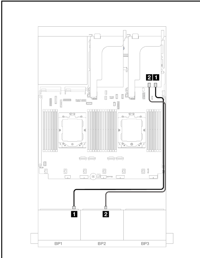
图 420. SAS/SATA 线缆布放
