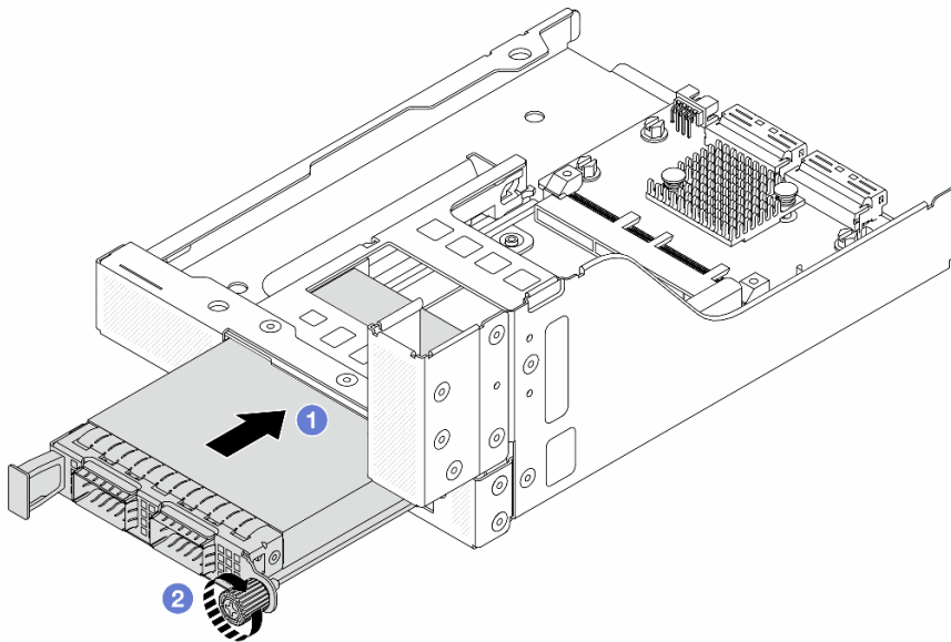
图 45. 安装 OCP 模块
