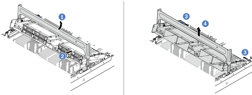
图 183. 卸下中间硬盘仓
