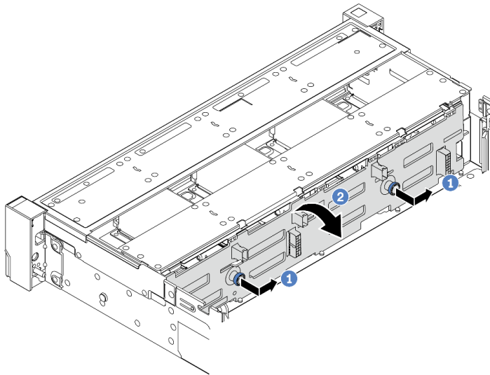
图 75. 卸下 3.5 英寸硬盘背板
