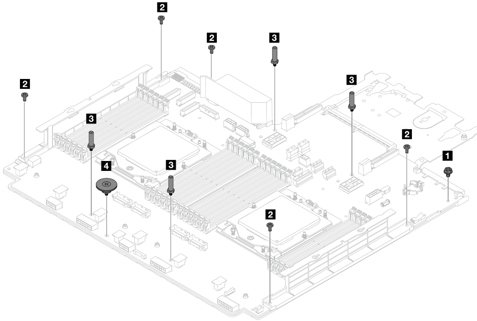
图 600. 从处理器板上卸下螺钉
