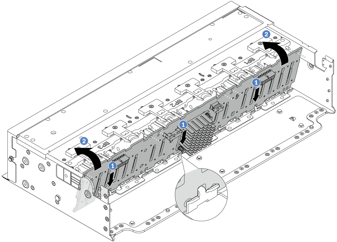
图 74. 安装 24 插槽扩展器背板
