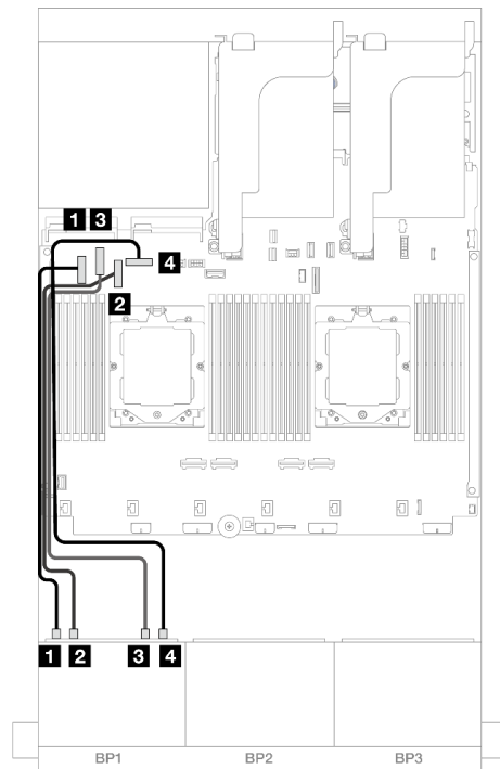
图 369. NVMe 线缆布放
