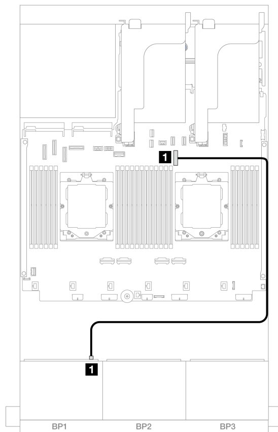
图 374. 到板载接口的 SAS/SATA 线缆布放
