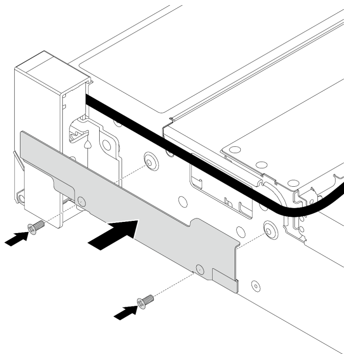
图 209. 安装线缆固定器
