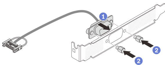
图 306. 组装串口模块
