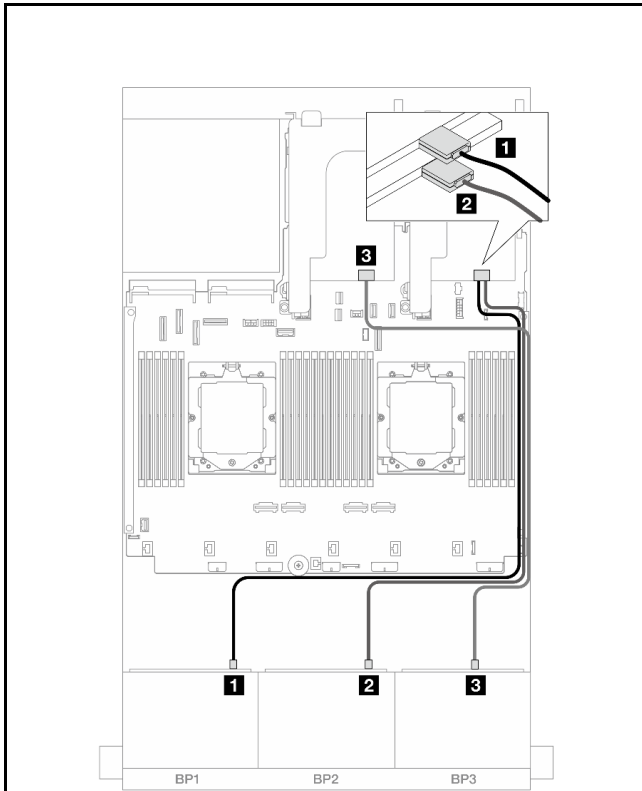
图 506. SAS/SATA 线缆布放
