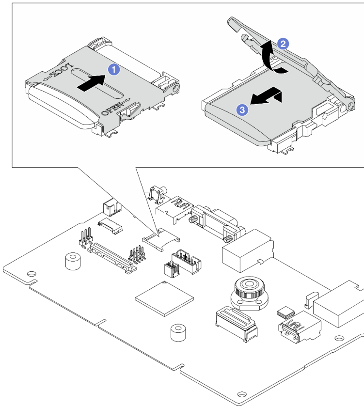
图 181. 卸下 MicroSD 卡
