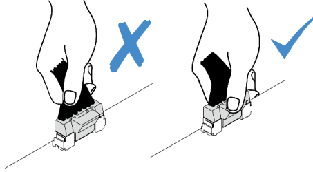
图 89. 从主板组合件上拔下线缆
