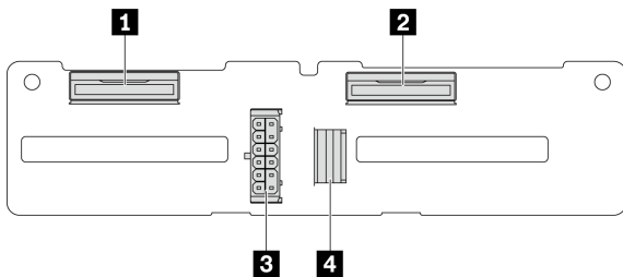
图 323. 4 x 2.5 英寸 AnyBay 背板接口
