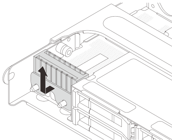
图 220. 取下橡胶
