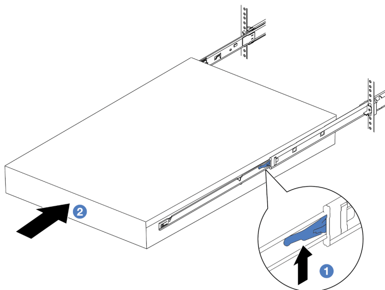
图 27. 将服务器装入机架
