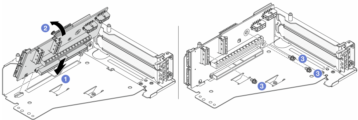
图 46. 安装转接卡
