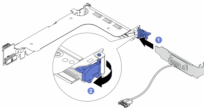
图 307. 安装串口模块
