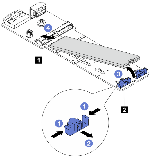
图 114. 卸下 M.2 硬盘
