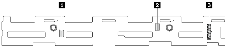
图 314. 8 x 3.5 英寸 SAS/SATA 背板接口
