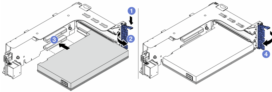
图 277. 将 PCIe 适配器安装到转接卡 1 或 2 组合件上
