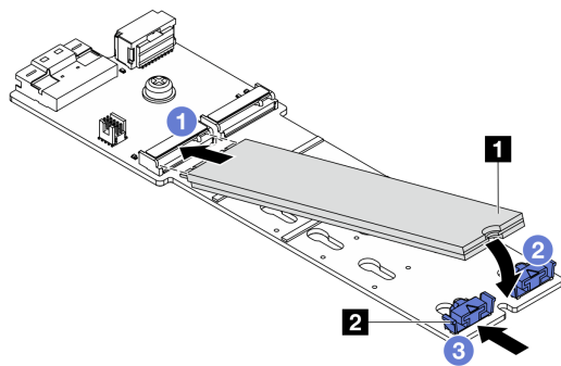
图 117. 安装 M.2 硬盘
