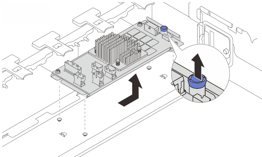
图 96. 卸下内部 CFF 适配器
