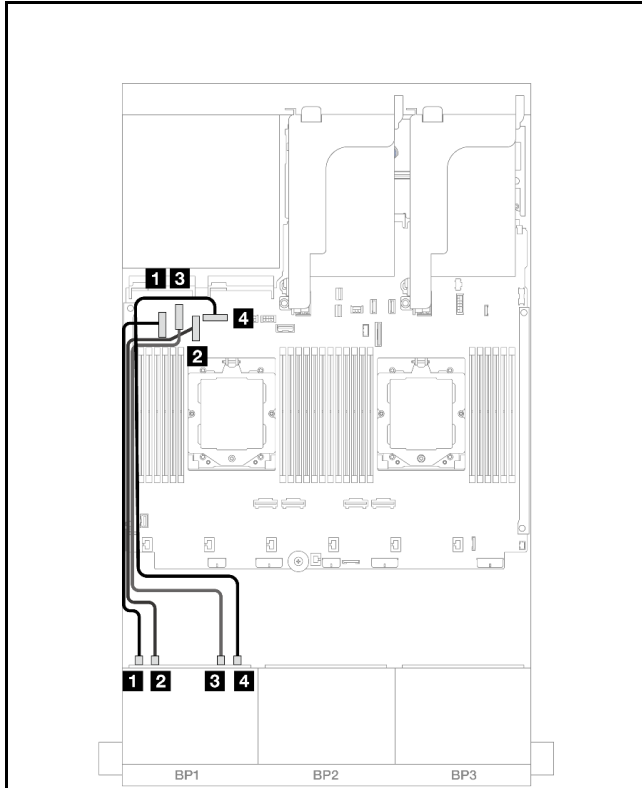
图 366. 装有两个处理器时的线缆布放
