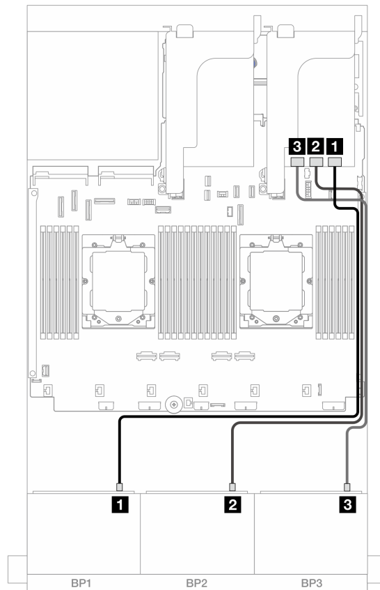
图 437. 到 32i 适配器的 SAS/SATA 线缆布放
