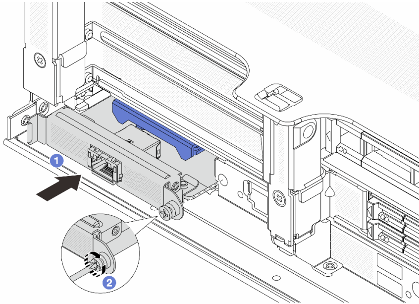
图 131. 安装管理 NIC 适配器
