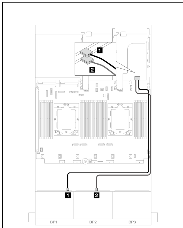
图 418. SAS/SATA 线缆布放
