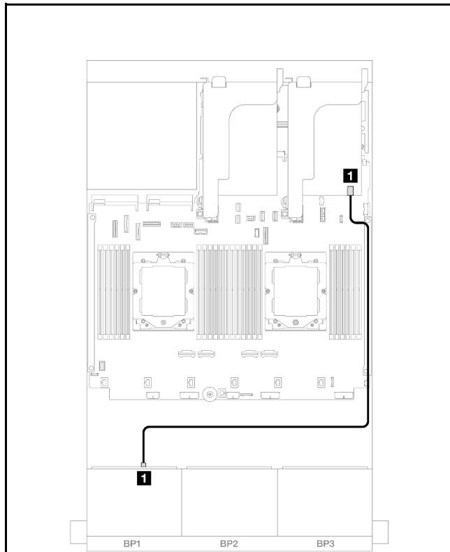
图 433. SAS/SATA 线缆布放
