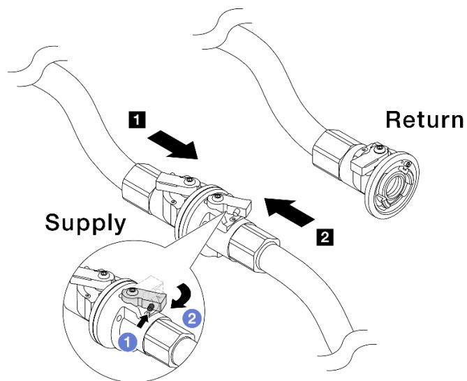
图 175. 设施供给侧到歧管供给侧
