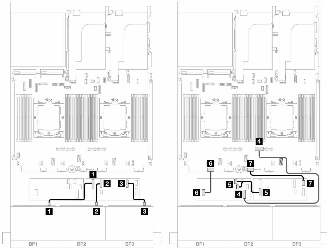
图 445. 到 CFF 扩展器和 CFF 16i 适配器的 SAS/SATA 线缆布放
