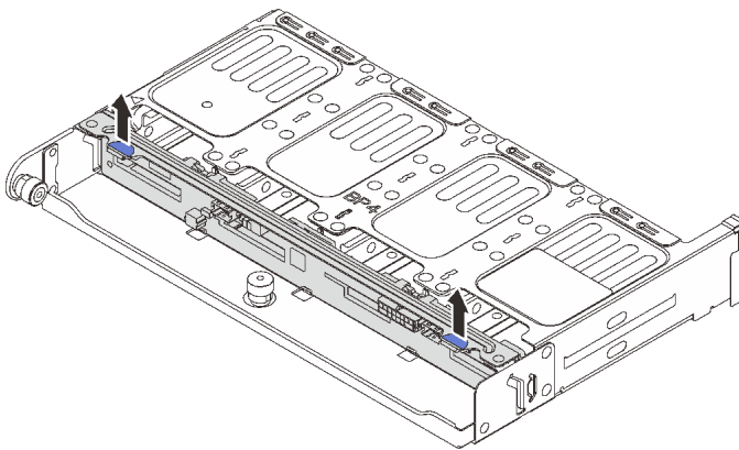
图 248. 卸下 8 x 2.5 英寸背面硬盘背板
