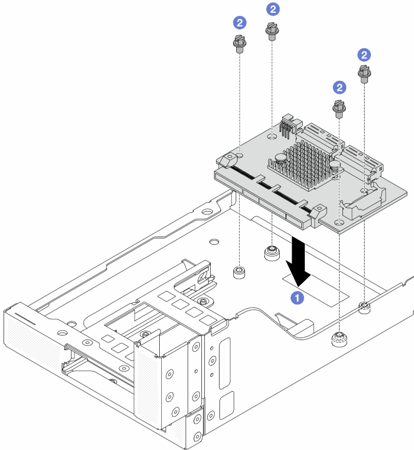
图 56. 安装正面 OCP 插转卡
