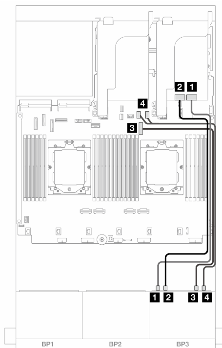
图 513. NVMe 线缆布放
