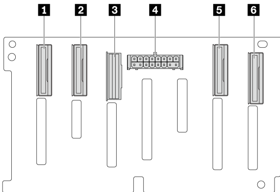
图 312. 8 x 2.5 英寸 AnyBay 背板接口
