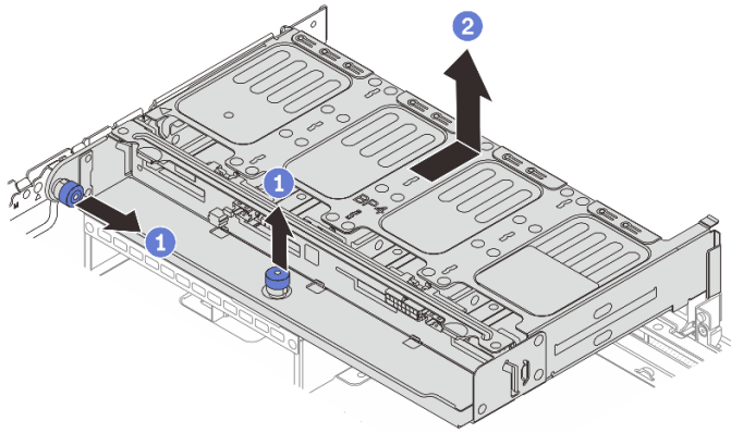
图 247. 卸下 8 x 2.5 英寸背面硬盘仓
