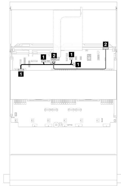
图 564. 中间/背面背板电源线布放
