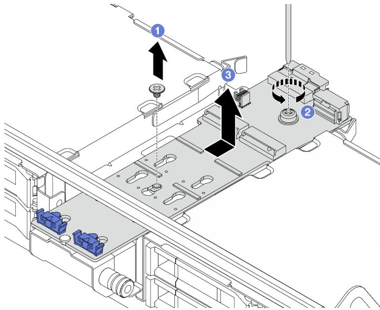
图 123. 从中间硬盘仓上卸下 M.2 背板
