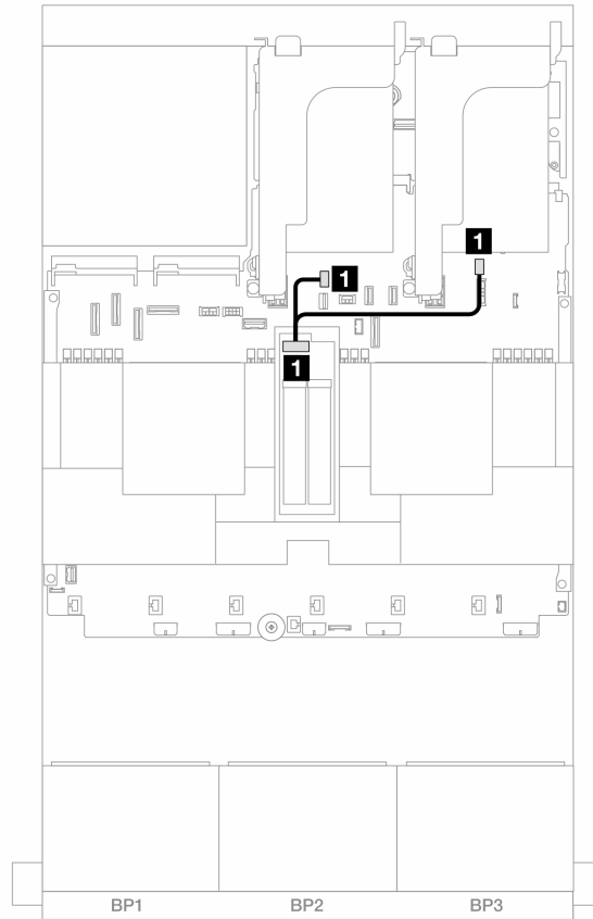
图 338. M.2 RAID SATA/NVME 2 插槽背板的线缆布放
