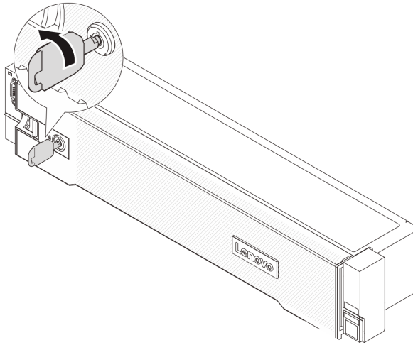
图 288. 锁定安全挡板
