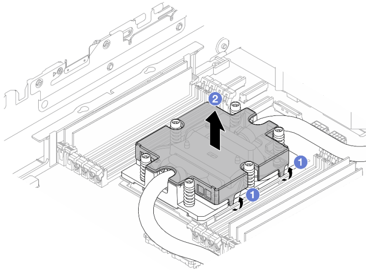
图 598. 卸下冷却板外盖
