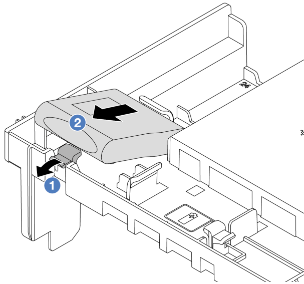
图 218. 从导风罩上卸下 RAID 快速充电模块
