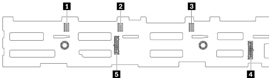
图 315. 12 x 3.5 英寸 SAS/SATA 背板接口
