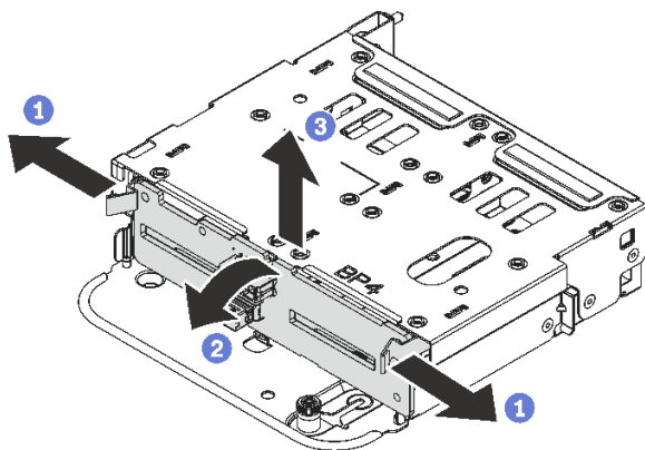
图 244. 卸下 4 x 2.5 英寸背面硬盘背板
