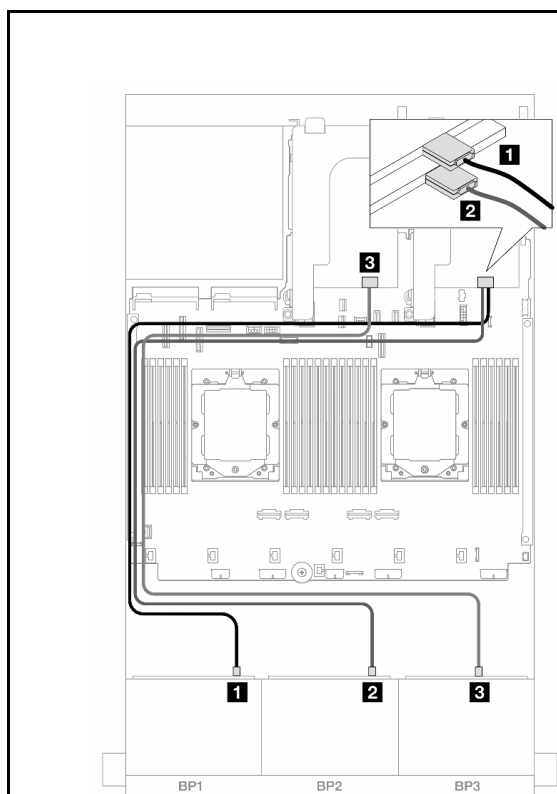
图 512. SAS/SATA 线缆布放
