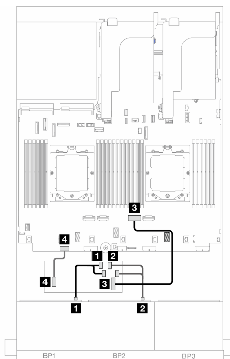
图 392. 装有一个处理器时的线缆布放
