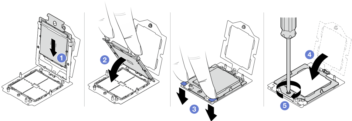
图 199. 安装处理器
