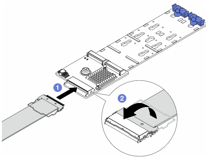
图 129. 将 M.2 线缆连接到 M.2 RAID SATA/NVME 2 插槽背板
