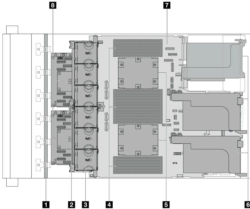
图 9. 带有标准散热器的俯视图
