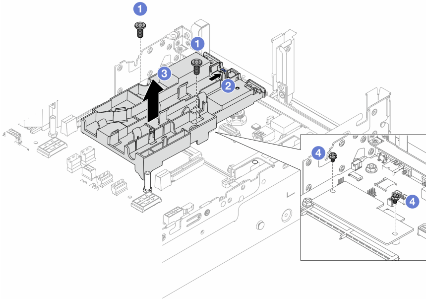
图 105. 卸下软管夹持器
