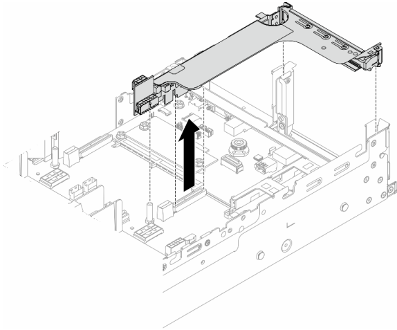
图 303. 卸下转接卡支架
