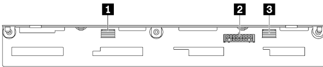
图 322. 8 x 2.5 英寸 SAS/SATA 背板接口
