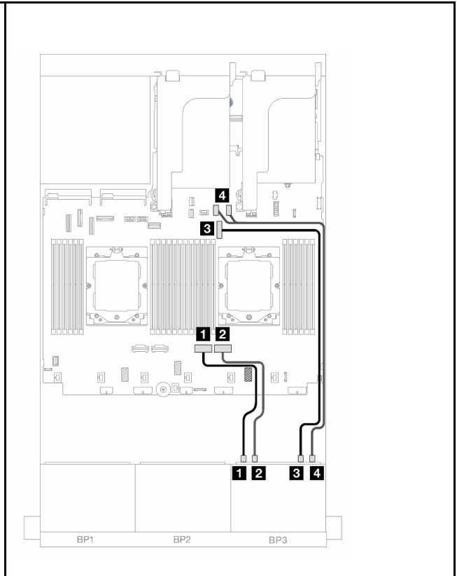
图 523. NVMe 线缆布放
