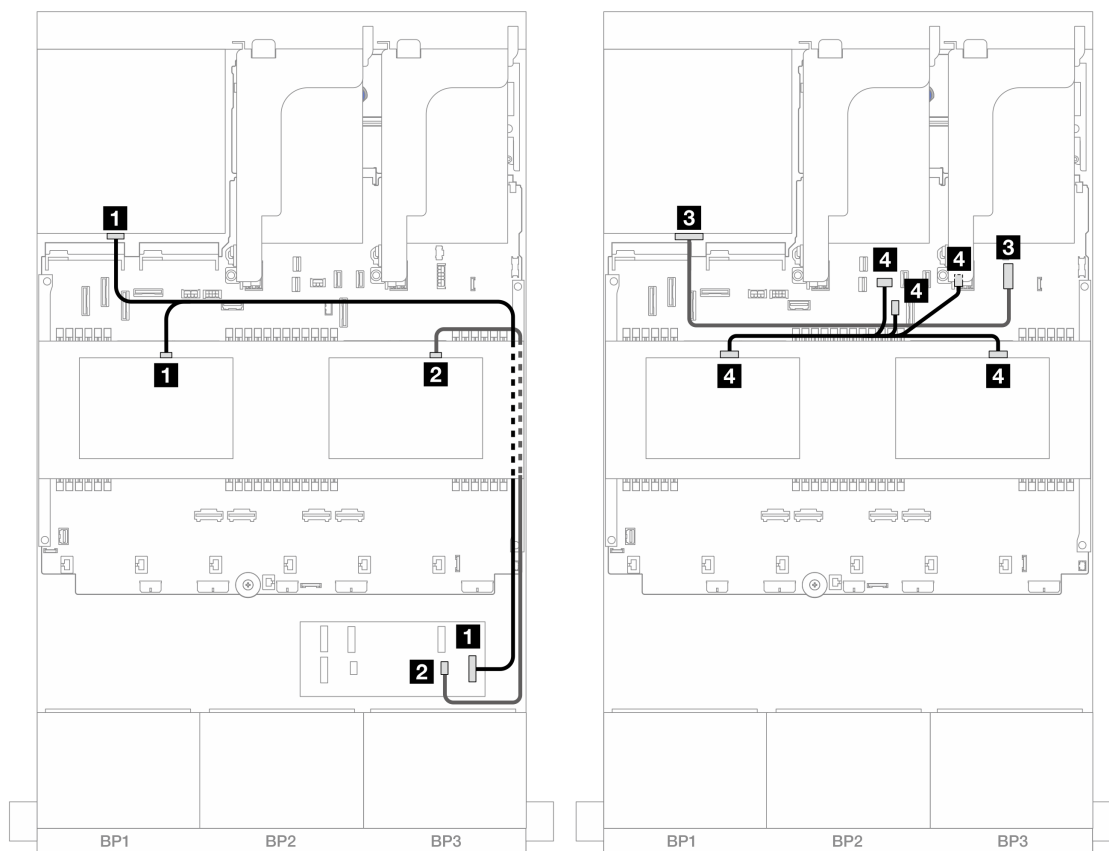
图 480. 中间/背面背板线缆布放
