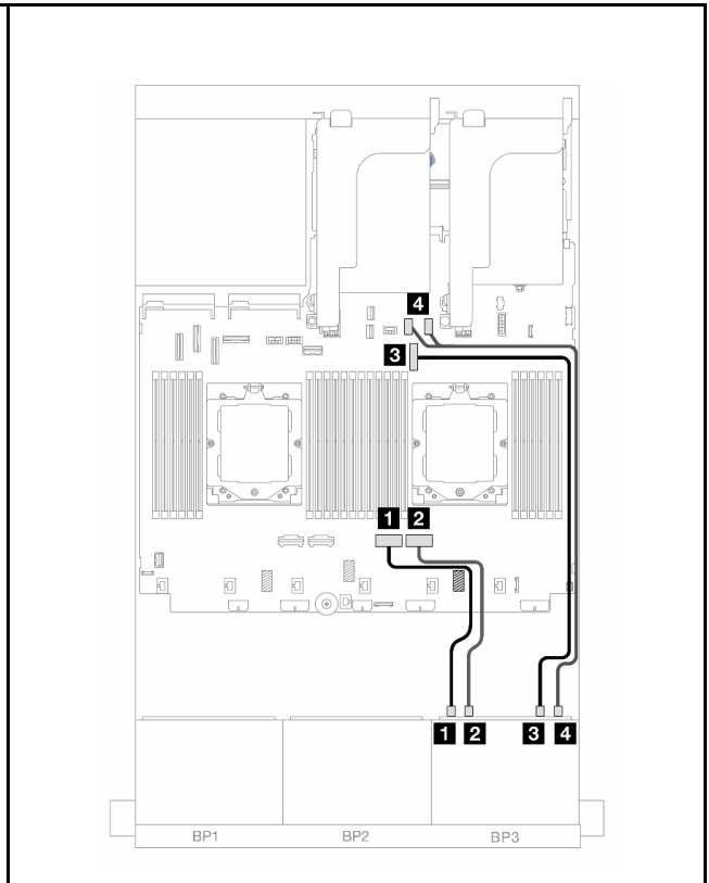
图 509. NVMe 线缆布放
