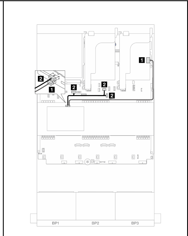
图 470. 中间背板线缆布放
