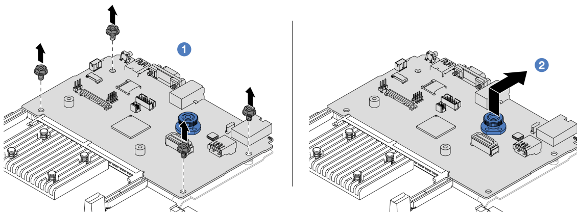
图 599. 将系统 I/O 板与处理器板分开
