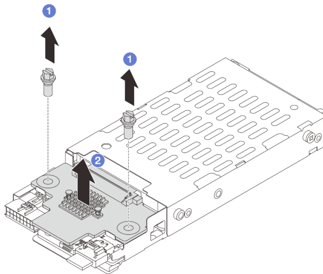
图 235. 卸下 7 毫米硬盘背板（顶部）
