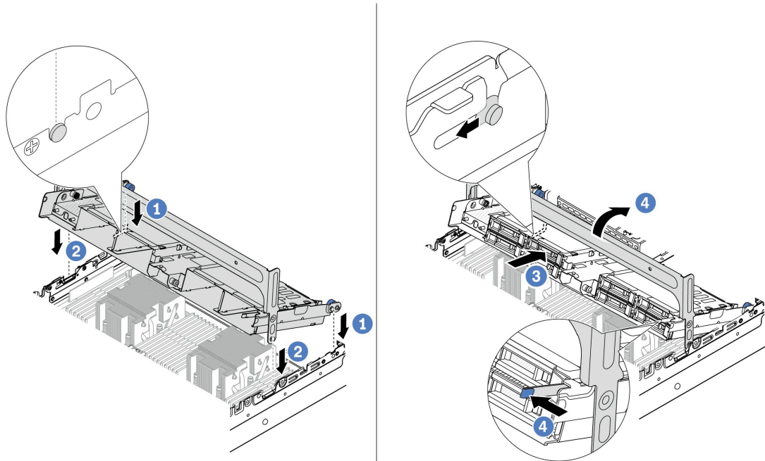
图 188. 安装中间硬盘仓和硬盘
