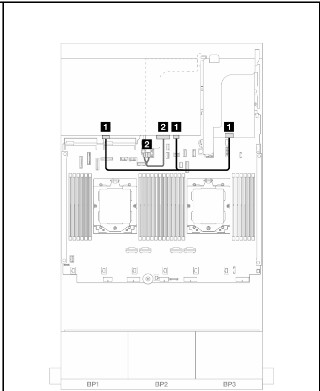
图 537. 背面背板线缆布放
