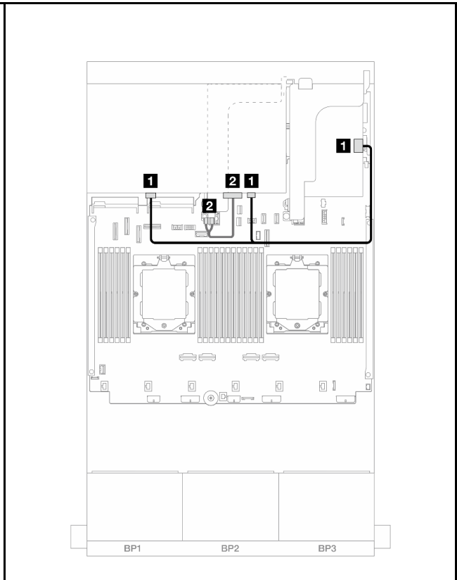
图 458. 背面背板线缆布放
