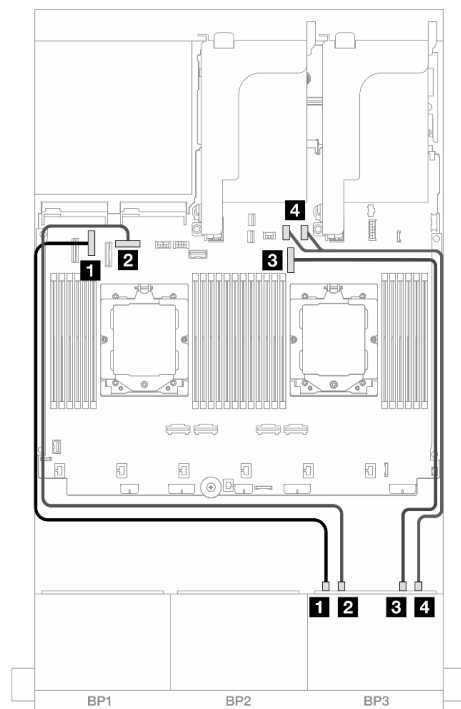
图 521. NVMe 线缆布放
