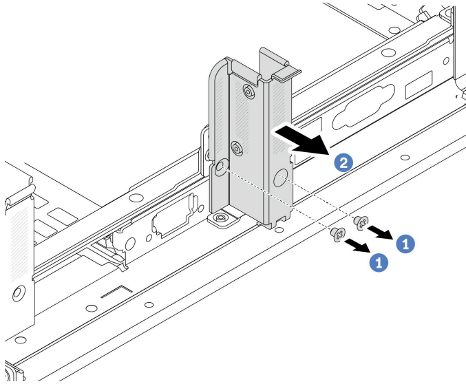
图 227. 卸下 B1 背面壁挂支架（中间）
