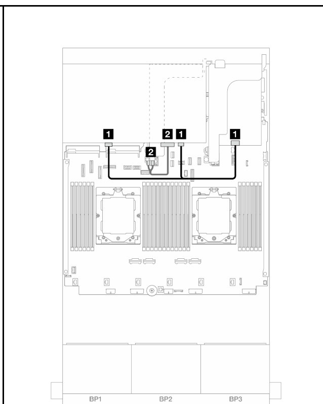
图 460. 背面背板线缆布放
