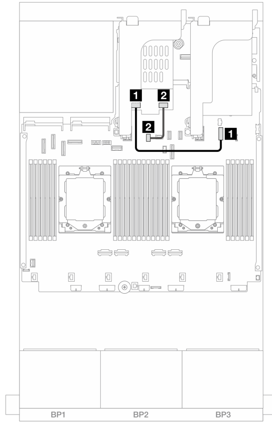
图 327. 7 毫米 RAID NVMe 2 插槽背板的线缆布放
