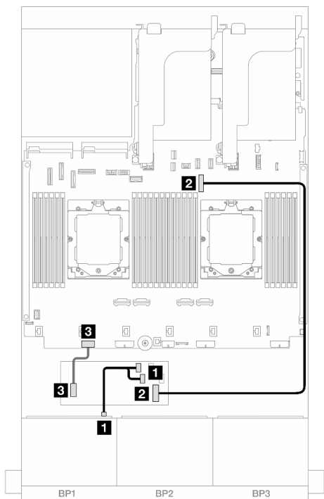
图 368. SAS/SATA 线缆布放
