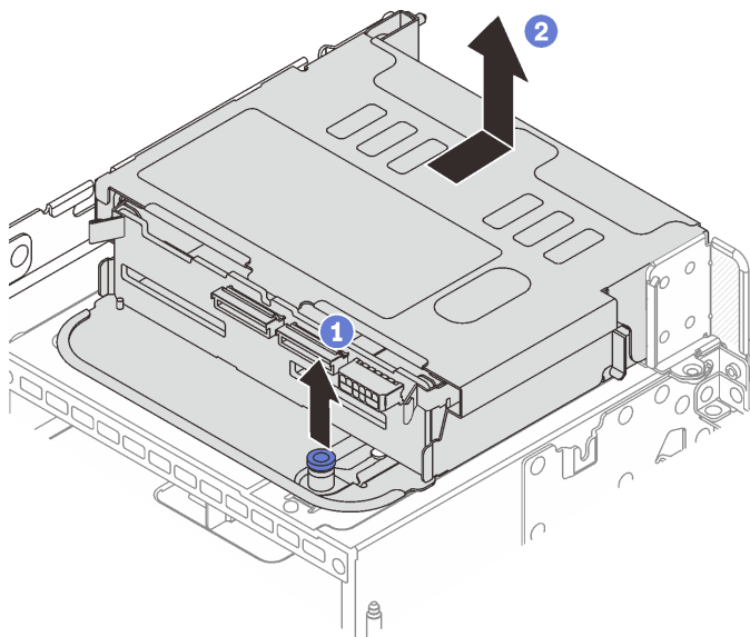
图 243. 卸下 4 x 2.5 英寸背面硬盘仓
