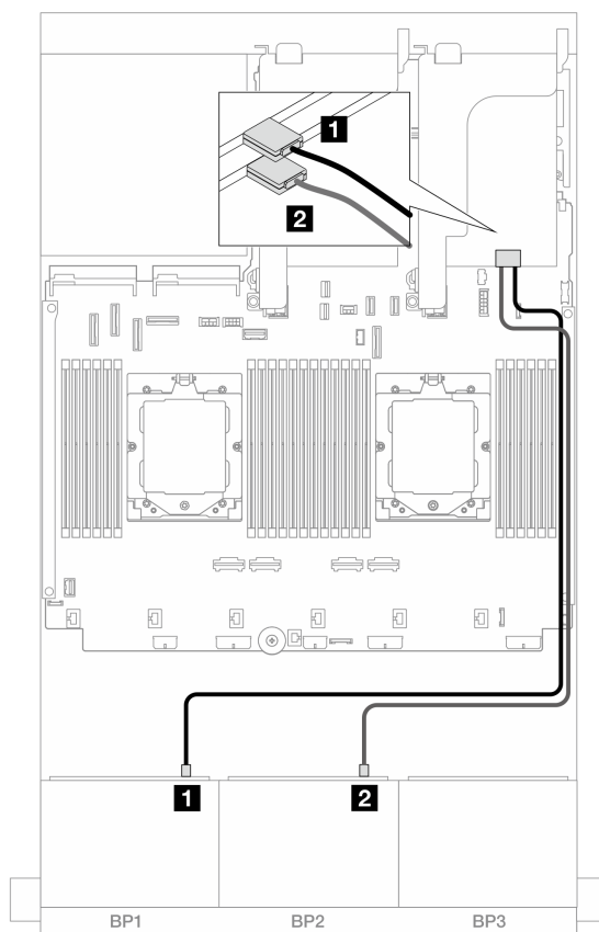
图 514. 到 8i 适配器的 SAS/SATA 线缆布放
