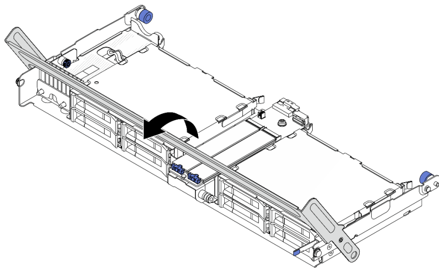
图 122. 打开中间硬盘仓的手柄
