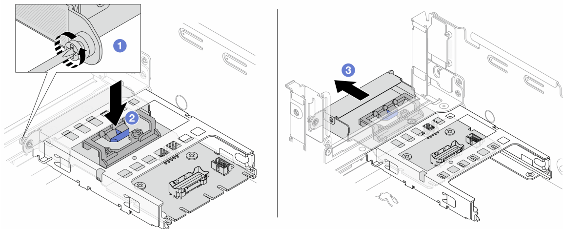
图 60. 卸下背面 OCP 插转卡
