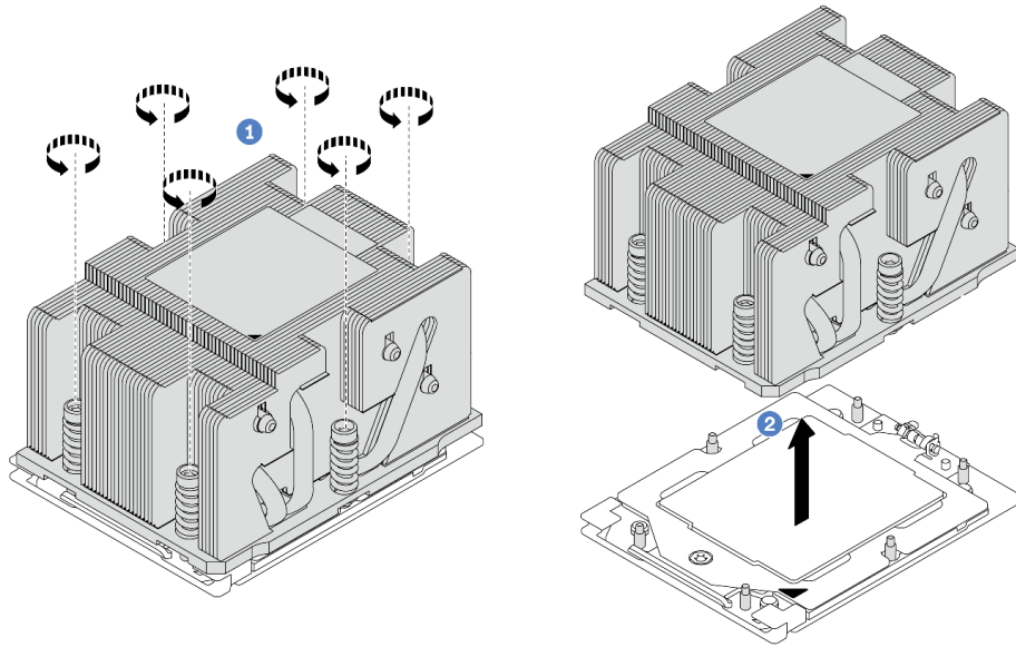
图 194. 卸下标准散热器
