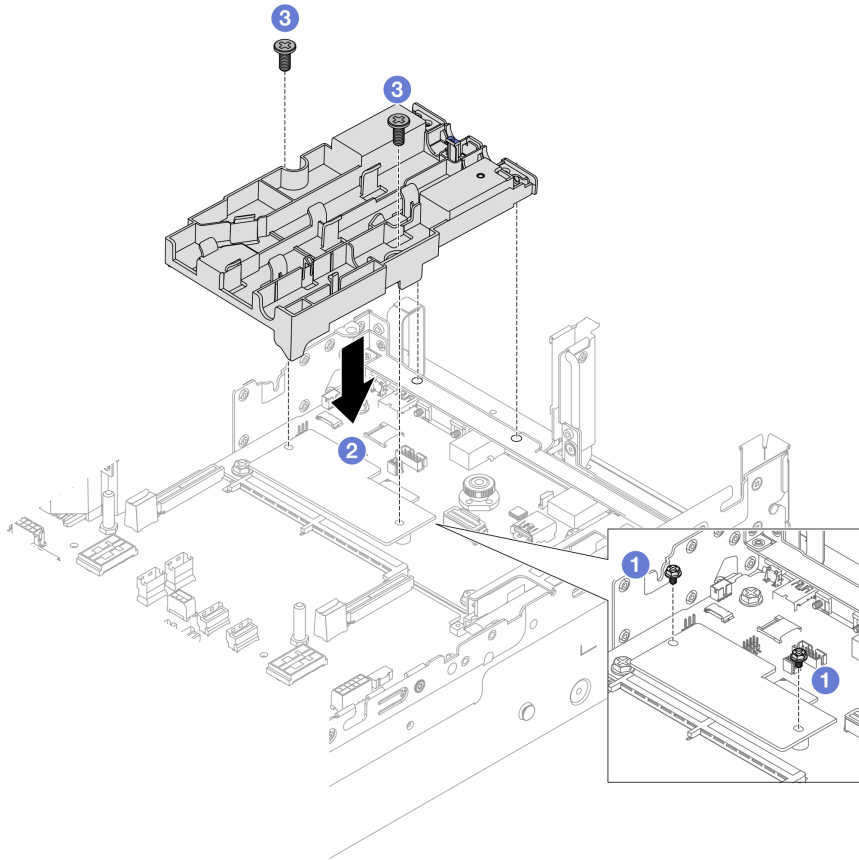
图 106. 安装软管夹持器
