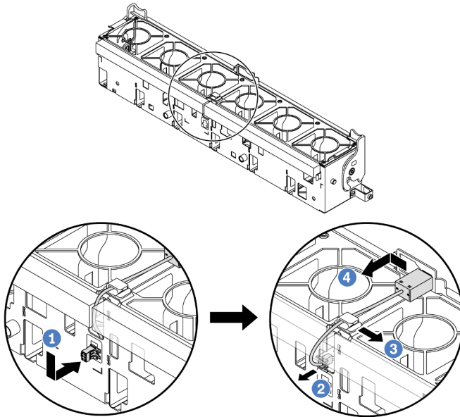
图 99. 卸下入侵感应开关
