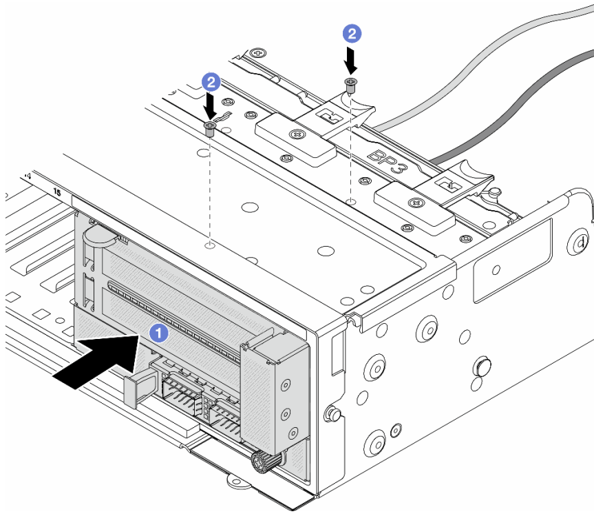
图 69. 安装正面适配器组合件
