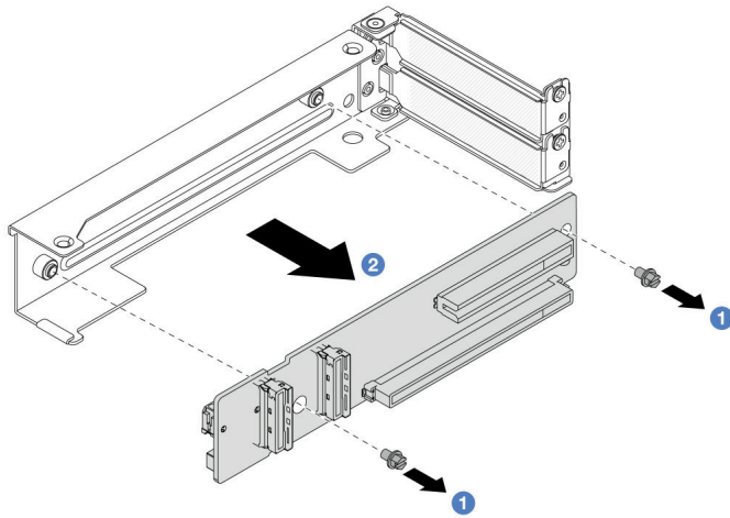
图 273. 从 4LP 转接卡 3/4 架上卸下转接卡
