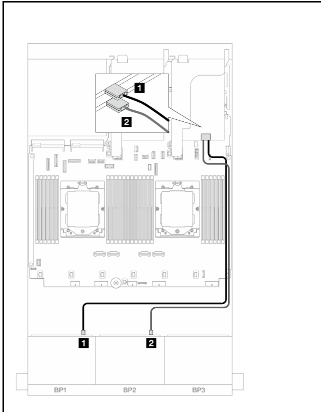
图 522. SAS/SATA 线缆布放
