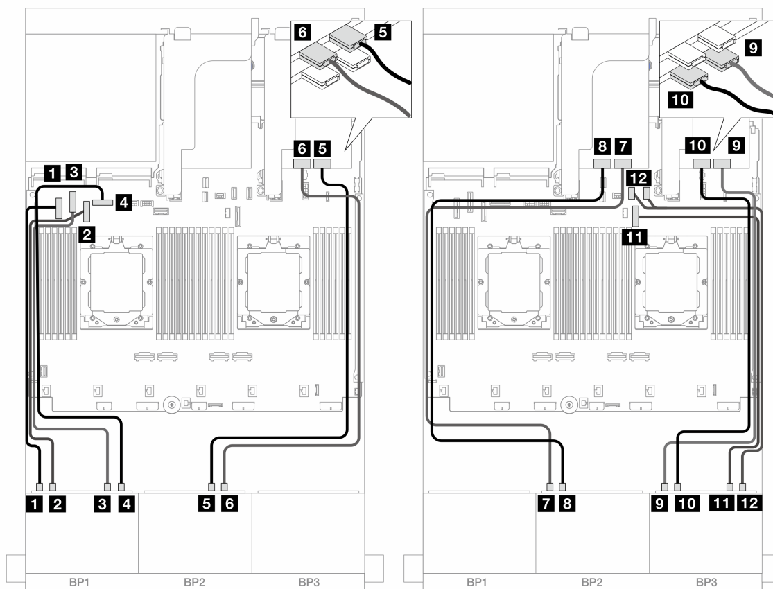
图 492. 到板载接口和重定时器卡的 NVMe 线缆布放
