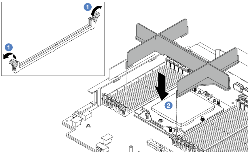
图 197. 安装处理器填充件
