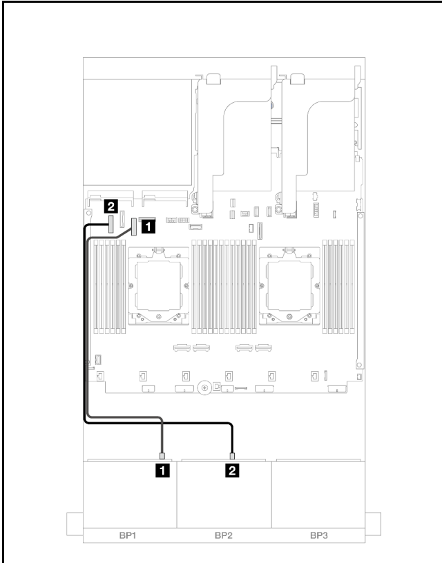
图 422. 装有两个处理器时的线缆布放
