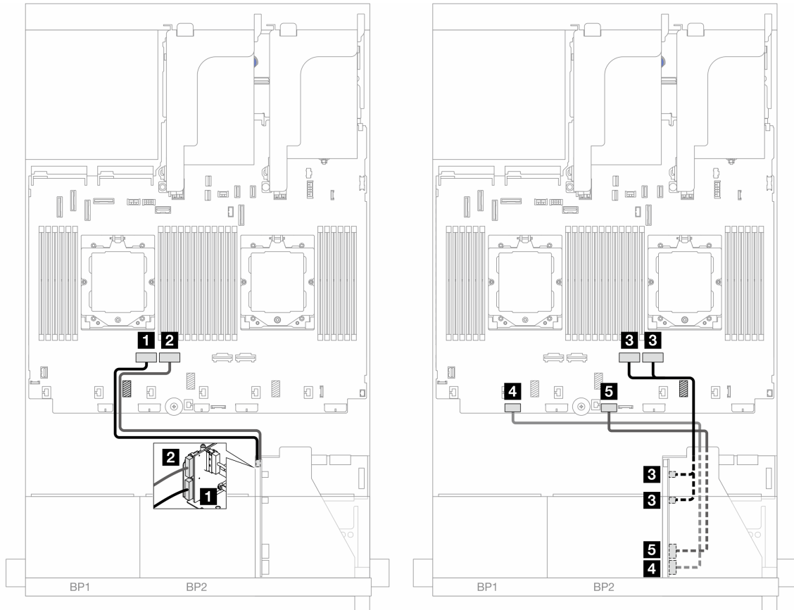
图 356. 带转接卡 3/4 的配置的线缆布放
