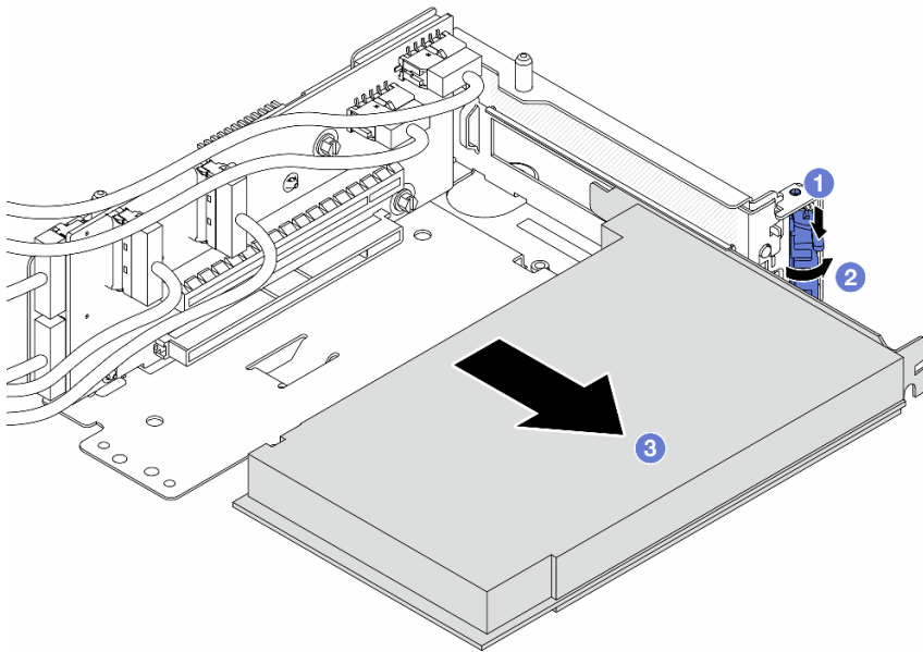
图 64. 从转接卡 5 架上卸下 PCIe 适配器
