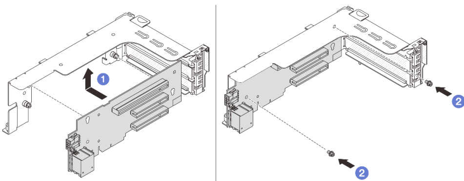
图 274. 将转接卡安装到转接卡 1 或 2 架上
