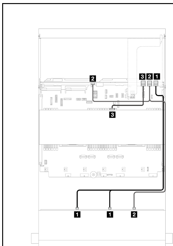
图 565. 正面/背面背板信号线缆布放
