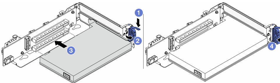
图 278. 将 PCIe 适配器安装到转接卡 3 组合件上
