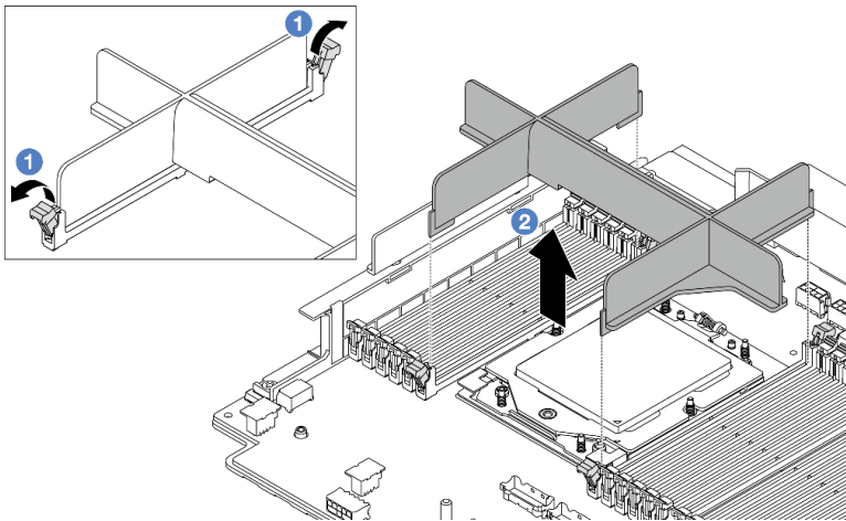
图 198. 卸下处理器填充件
