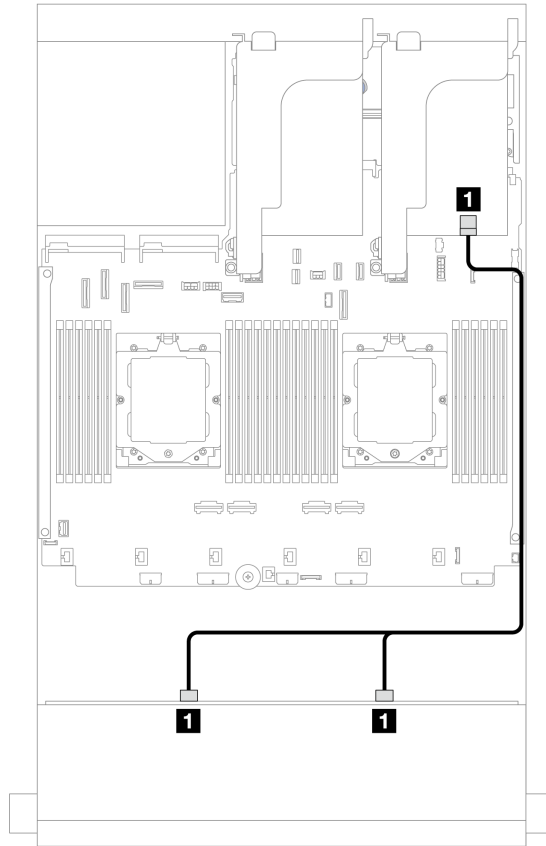
图 543. 到 8i RAID/HBA 适配器的线缆布放
