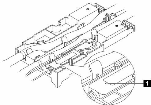
图 596. 漏液检测传感器模块上的 LED
