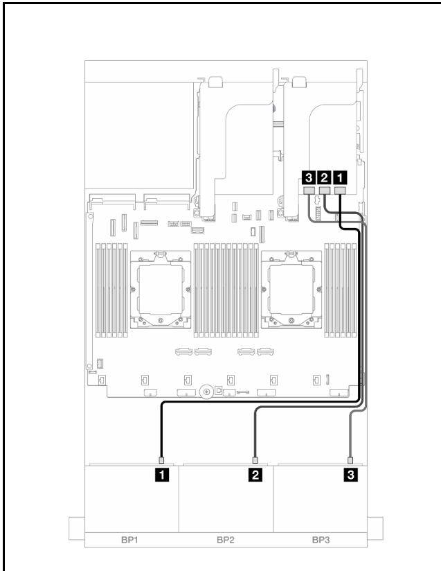
图 457. 正面背板线缆布放
