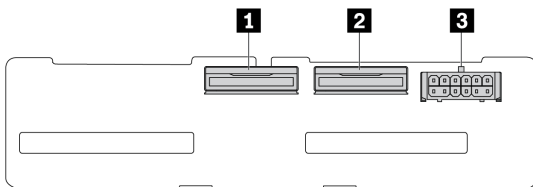
图 319. 4 x 2.5 英寸 NVMe 背板接口
