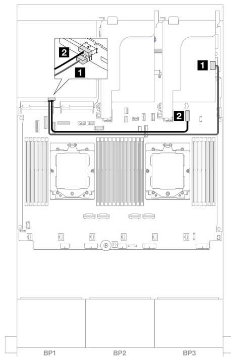
图 441. 背面背板线缆布放
