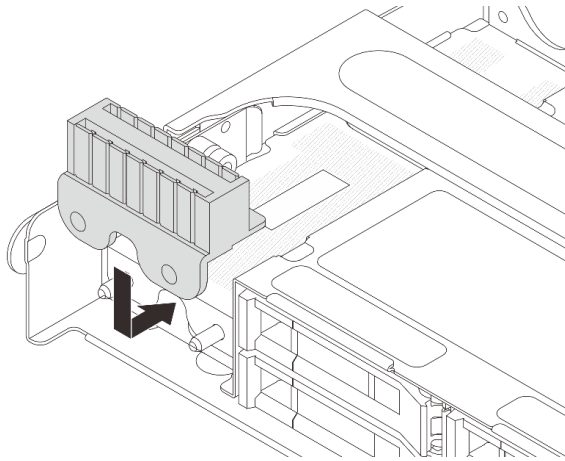
图 225. 安装橡胶
