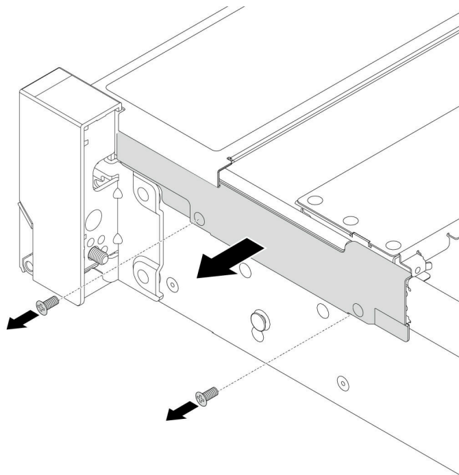
图 204. 卸下线缆固定器
