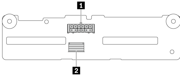
图 318. 4 x 2.5 英寸 SAS/SATA 背板接口
