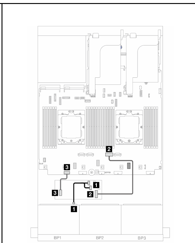
图 364. 装有一个处理器时的线缆布放
