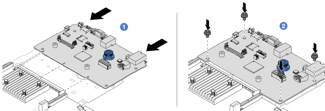
图 296. 将系统 I/O 板安装到处理器板上
