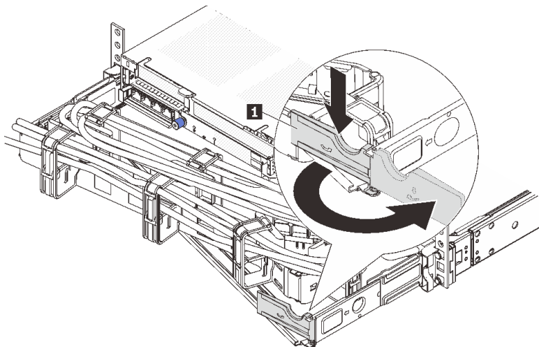
图 189. 调整 CMA
