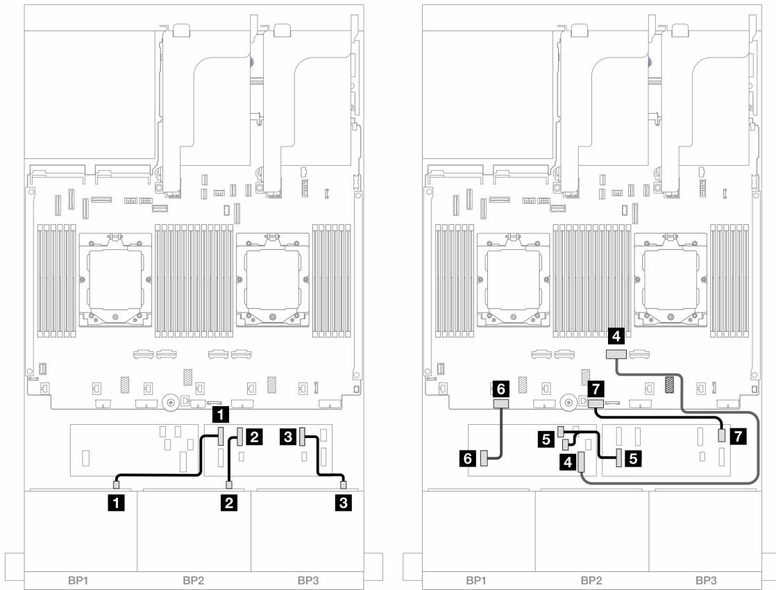
图 454. 到 CFF 扩展器和 CFF 16i 适配器的 SAS/SATA 线缆布放
