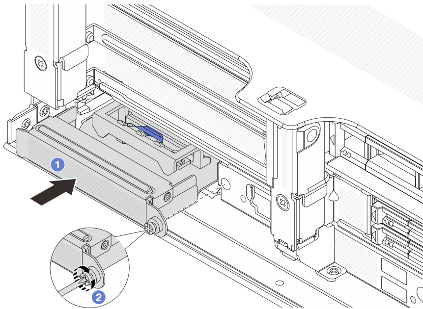
图 61. 安装背面 OCP 插转卡
