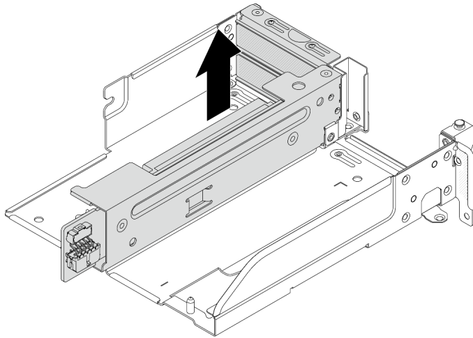
图 266. 卸下转接卡 3/4 组合件
