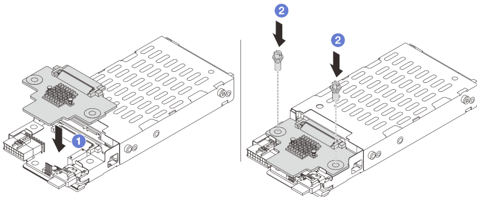
图 238. 安装 7 毫米硬盘背板（顶部）
