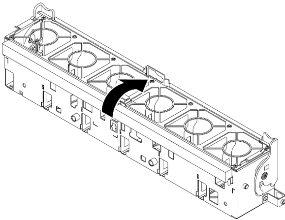
图 98. 旋转风扇架
