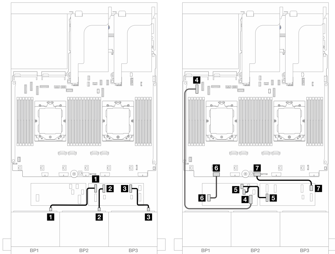
图 486. 到 CFF 扩展器和 CFF 16i 适配器的 SAS/SATA 线缆布放
