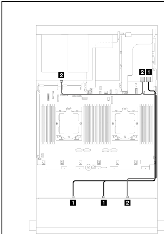
图 551. 正面/背面背板信号线缆布放
