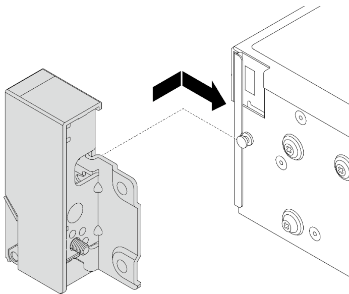
图 207. 安装机架滑锁
