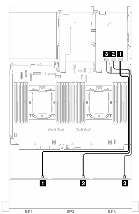
图 473. 正面背板线缆布放
