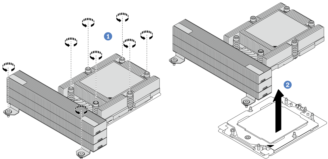
图 195. 卸下高性能散热器
