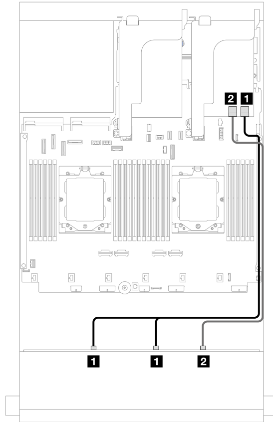
图 560. 到 16i RAID/HBA 适配器的线缆布放
