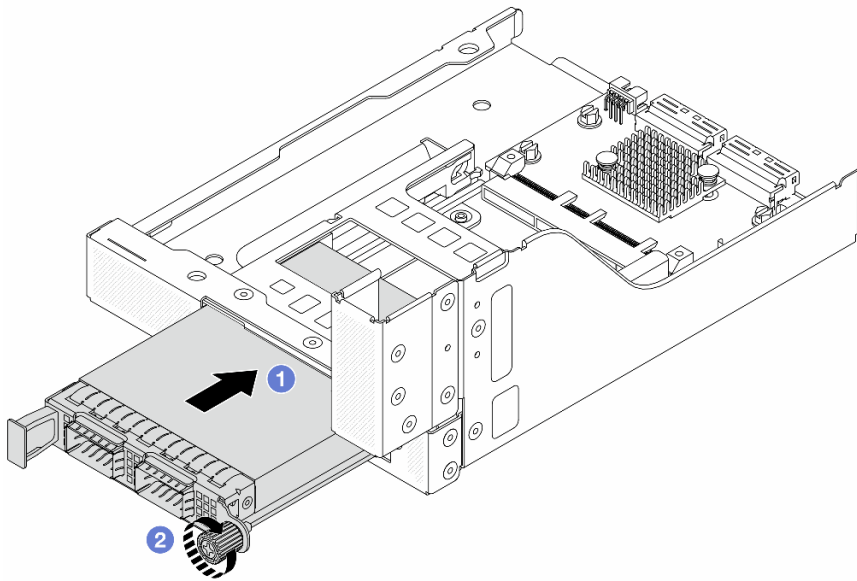
图 57. 安装 OCP 模块
