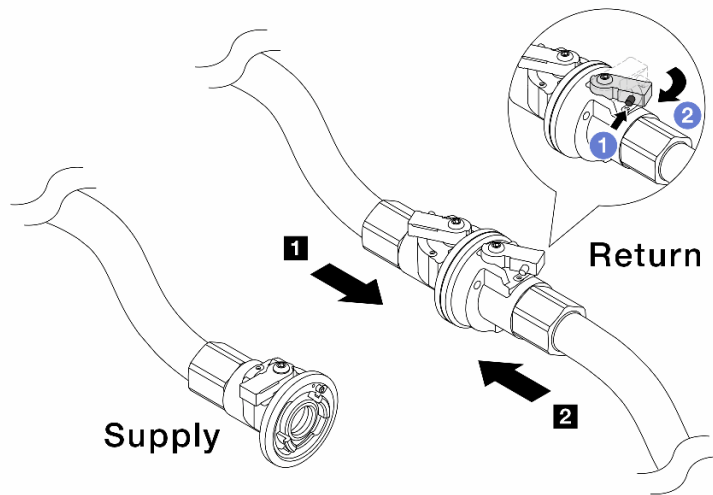
图 172. 设施供给侧到歧管回流侧
