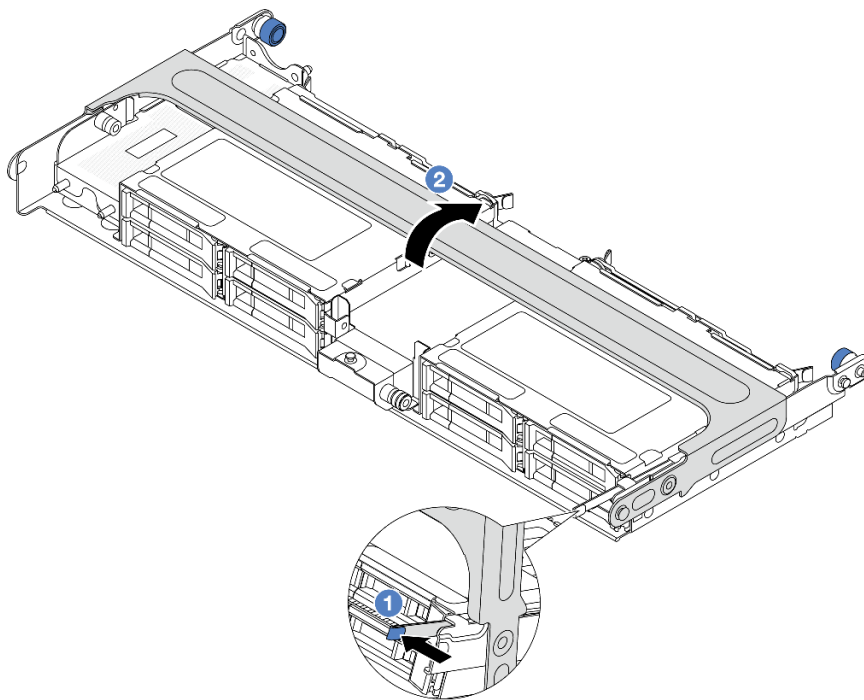
图 224. 合上中间硬盘仓的手柄
