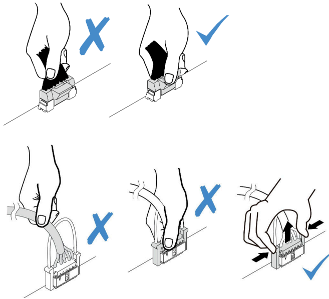
图 203. 从主板组合件上拔下线缆
