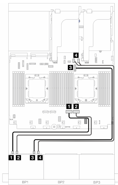
图 385. 装有一个处理器时的线缆布放
