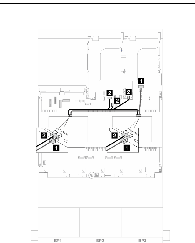
图 476. 中间背板线缆布放
