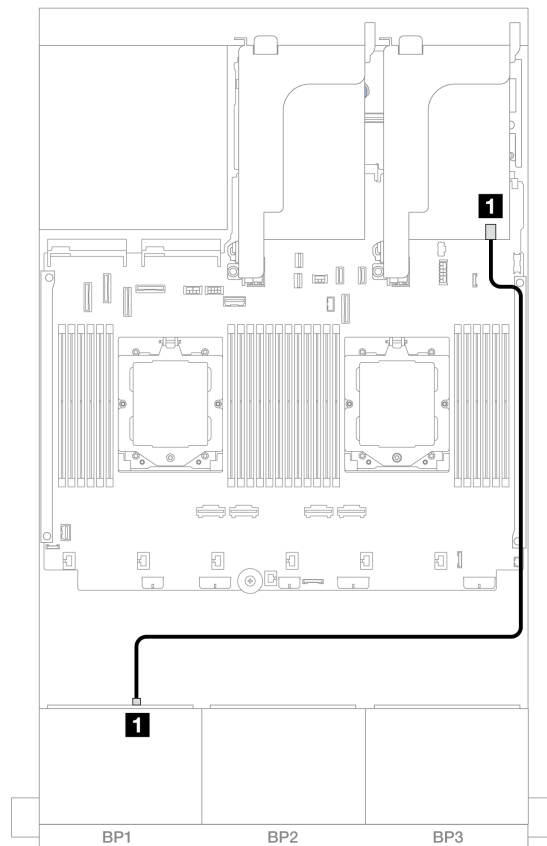
图 365. 到 8i/16i RAID/HBA 适配器的 SAS/SATA 线缆布放
