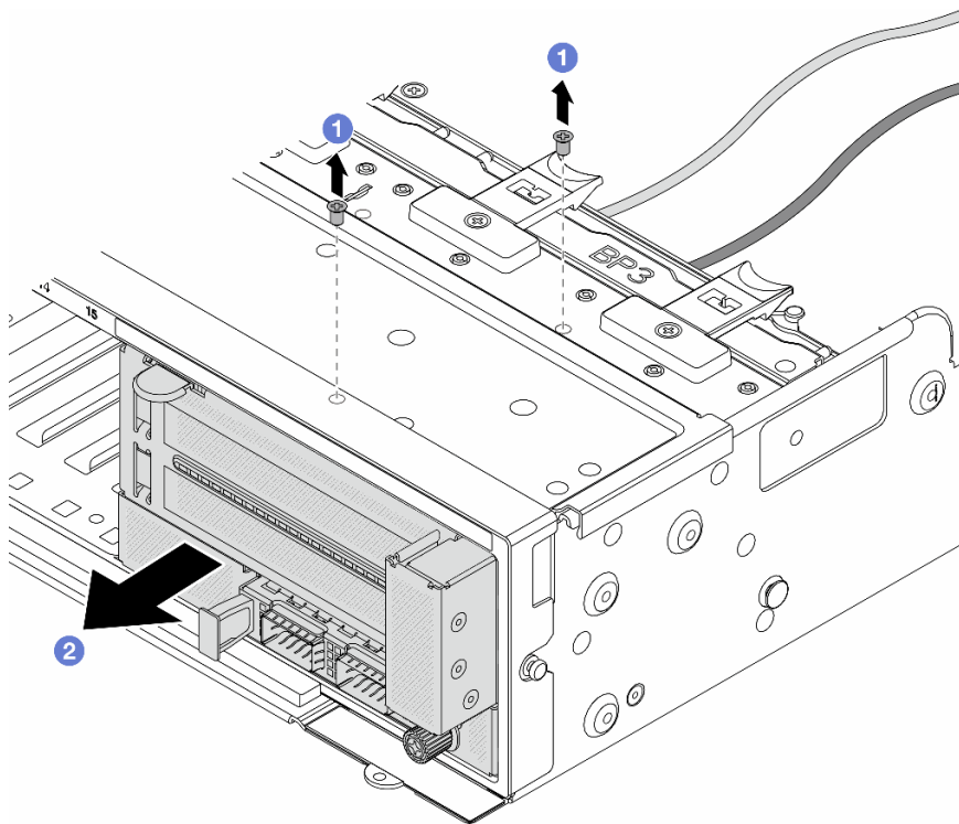
图 52. 卸下正面适配器组合件
