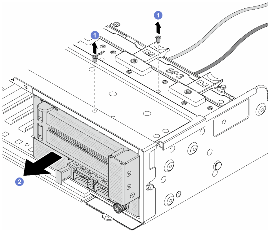
图 62. 卸下正面适配器组合件
