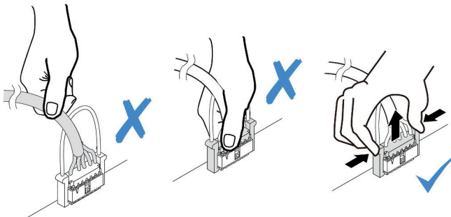
图 302. 从系统 I/O 板上拔下线缆
