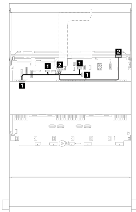
图 566. 背面背板电源线布放
