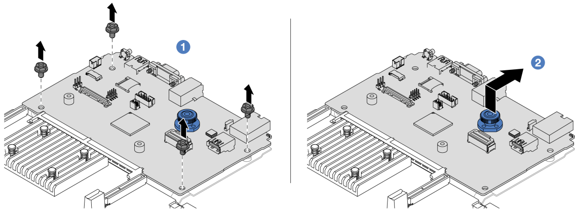
图 293. 将系统 I/O 板与处理器板分开
