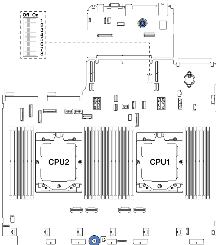
圖例 13. 主機板組件上的開關區塊
