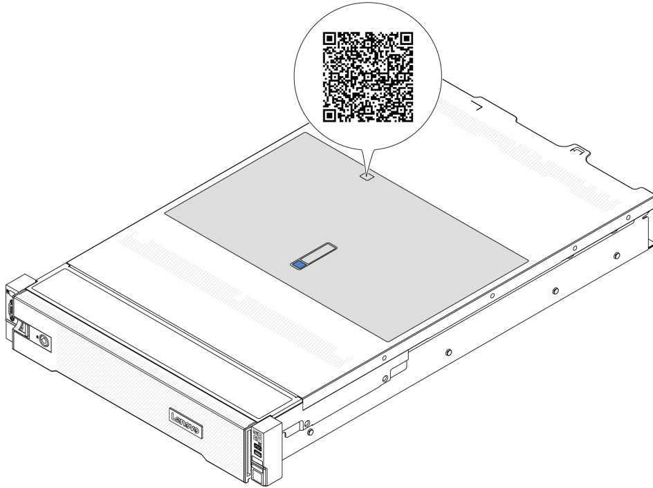
圖例 25. 服務標籤和 QR 代碼
