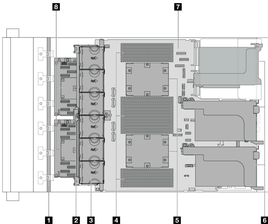
圖例 9. 配備標準散熱槽的俯視圖
