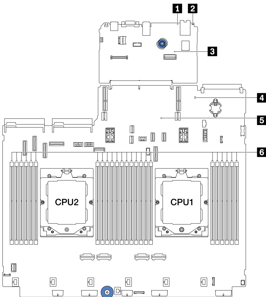
圖例 19. 主機板組件 LED
