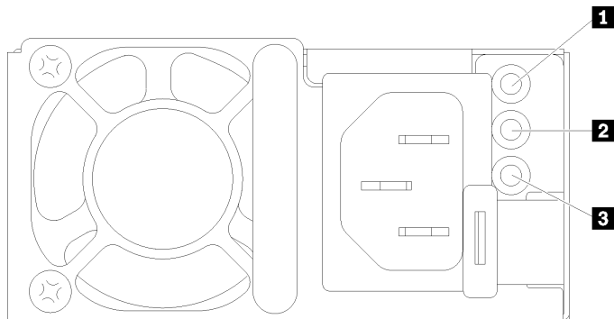
圖例 18. 電源供應器 LED
