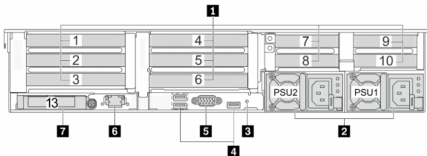
配備十個 PCIe 插槽的背面圖
