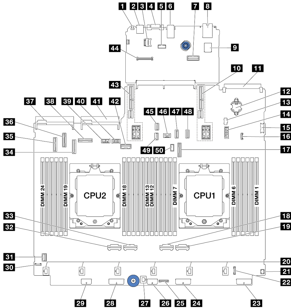
圖例 12. 主機板組件接頭
