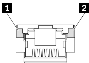
圖例 17. XCC 系統管理埠 LED
