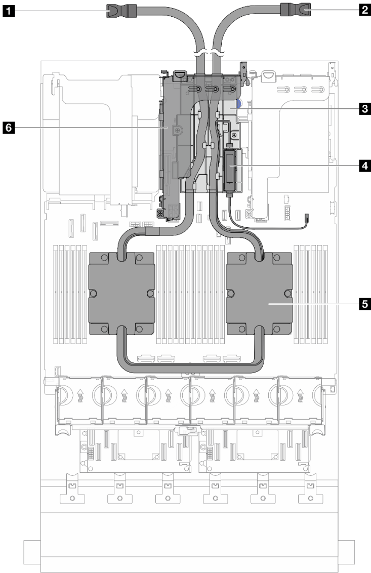
圖例 10. DWCM 的俯視圖
