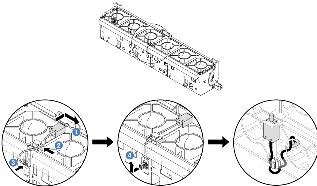
圖例 100. 安裝入侵開關
