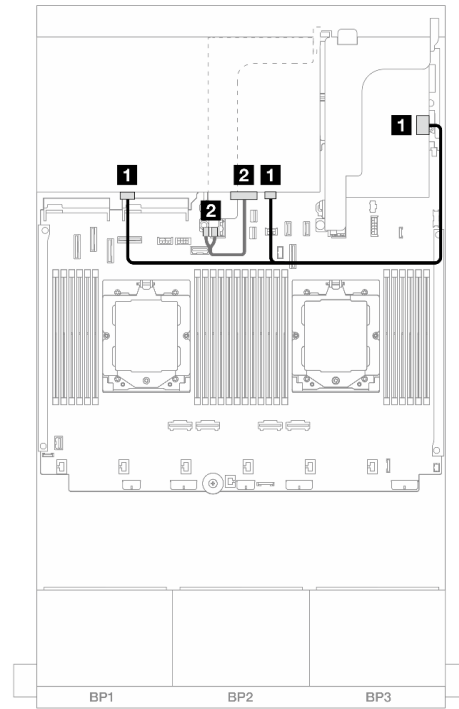
圖例 458. 後方背板纜線佈線
