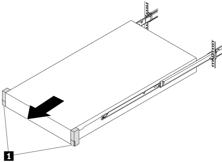
圖例 21. 拉出伺服器
