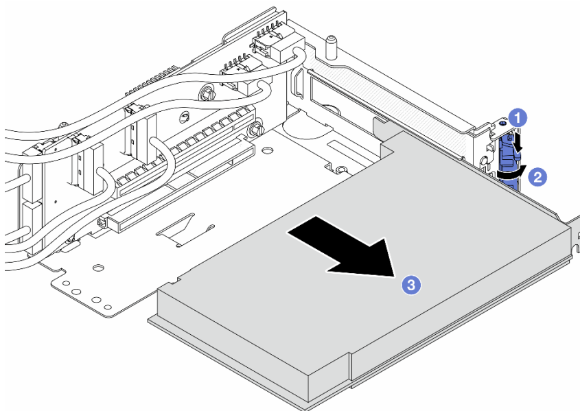
圖例 40. 從擴充卡 5 匣卸下 PCIe 配接卡
