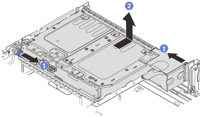
圖例 251. 卸下 2 x 3.5 吋背面框架
