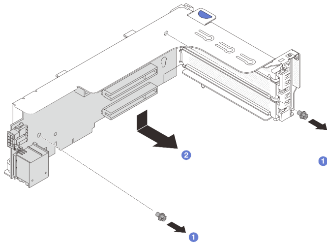
圖例 271. 從擴充卡 1 匣或擴充卡 2 匣卸下擴充卡
