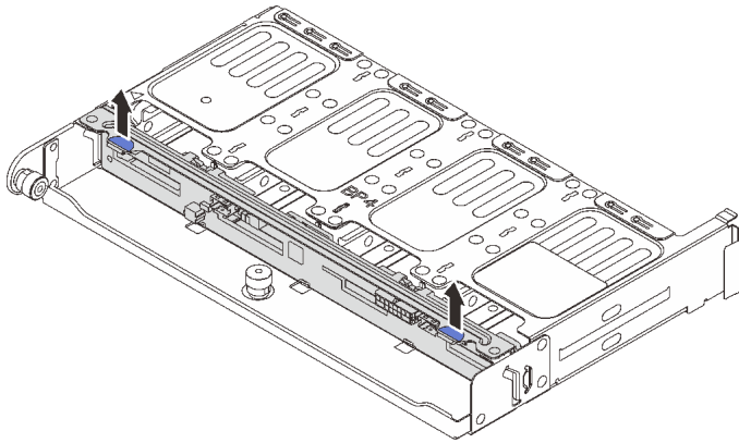
圖例 248. 卸下後方 8 x 2.5 吋硬碟背板
