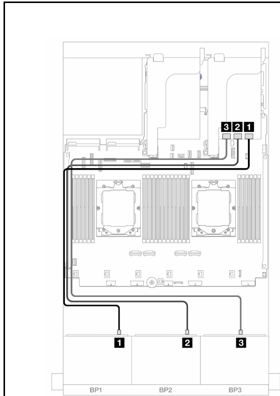
圖例 510. SAS/SATA 纜線佈線
