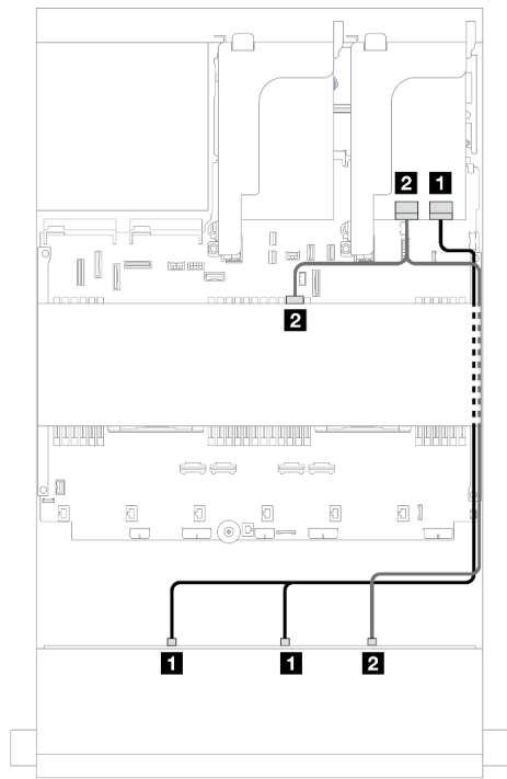
圖例 558. 前方/中間背板信號線佈線
