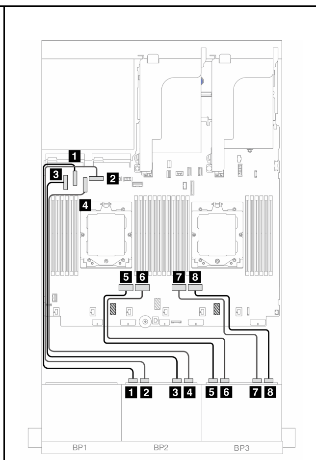
圖例 500. NVMe 纜線佈線
