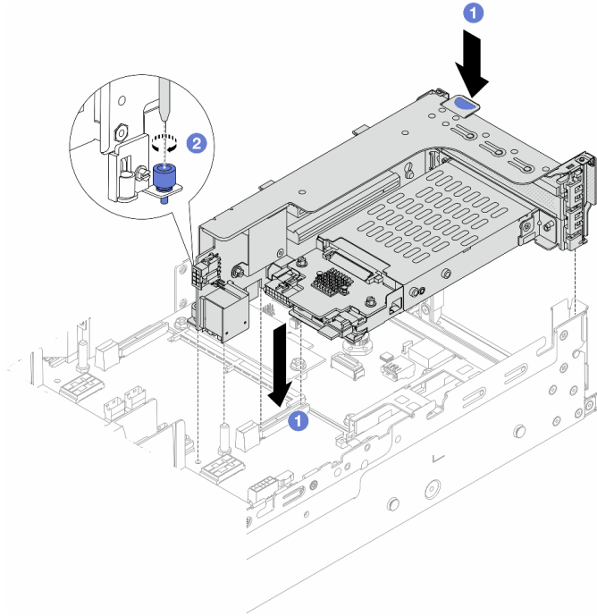
圖例 241. 安裝 2FH + 7 公釐 SSD 擴充卡匣
