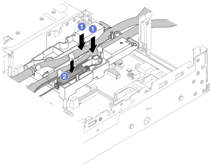
圖例 110. 放置水管和模組
