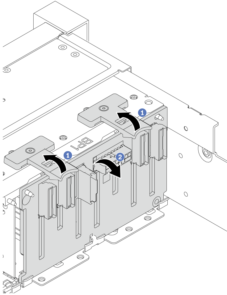
圖例 70. 卸下 8 機槽硬碟背板
