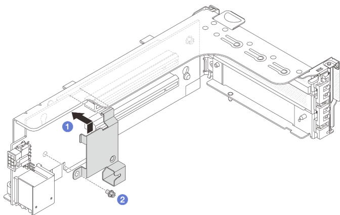
圖例 239. 安裝 7 公釐框架固定夾
