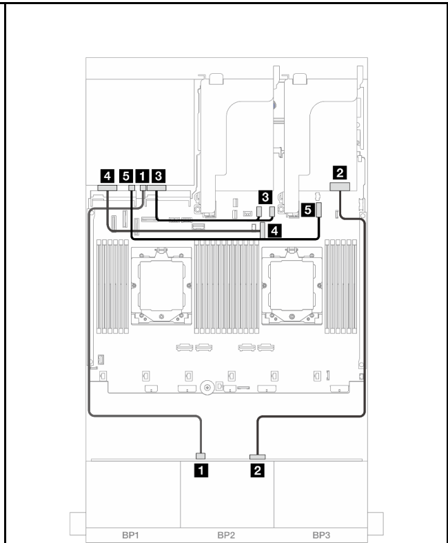
圖例 535. 安裝了一個處理器的纜線佈線
