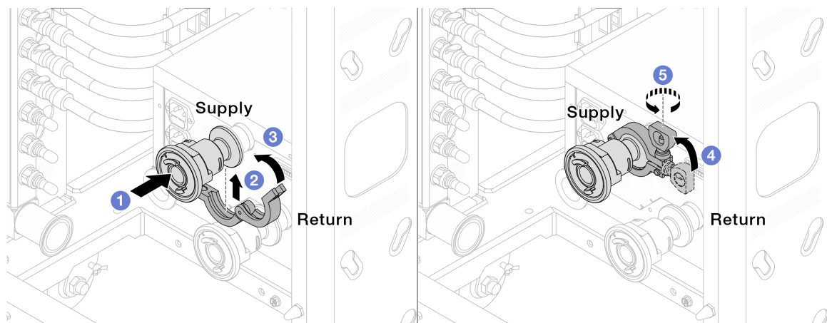
圖例 148. 安裝球閥
