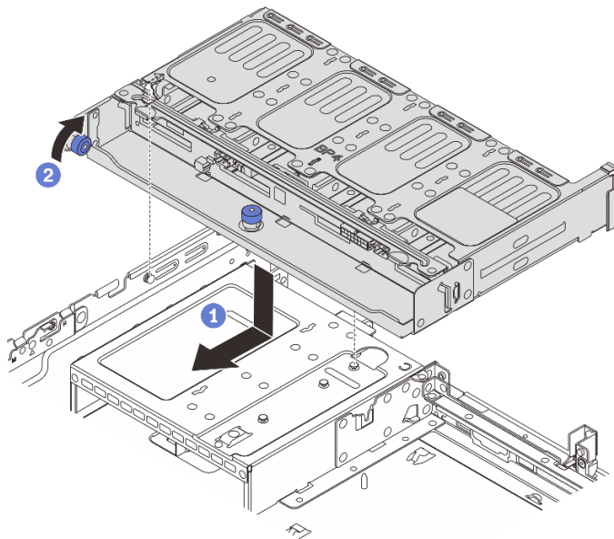
圖例 250. 安裝 8 x 2.5 吋背面框架
