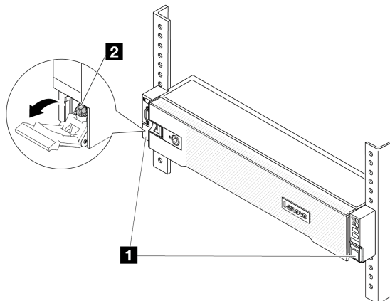
圖例 29. 將伺服器固定到機架正面
