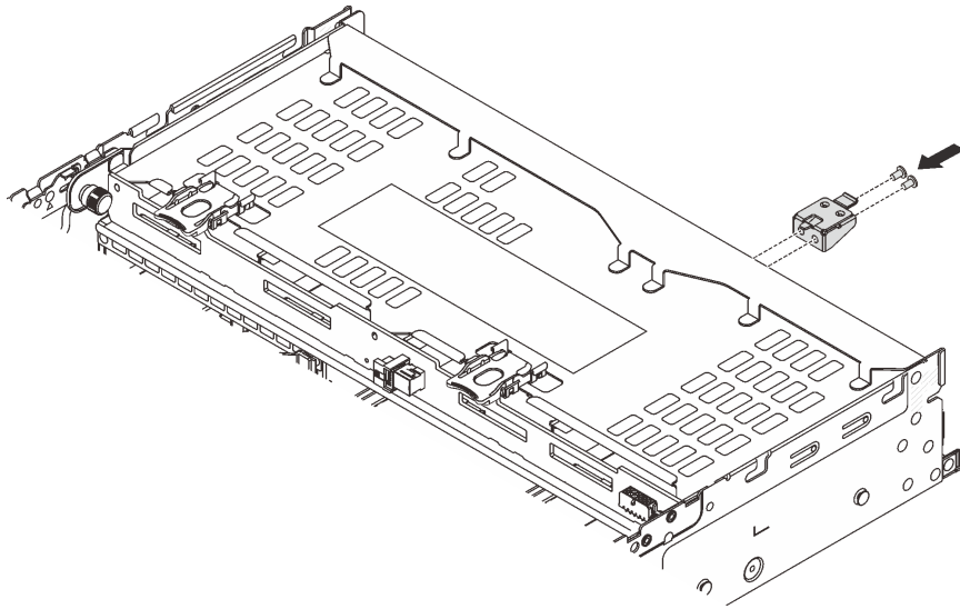
圖例 259. 安裝上蓋支撐托架
