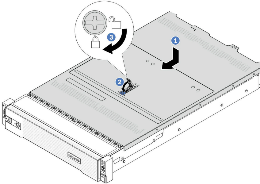
圖例 310. 安裝上蓋
