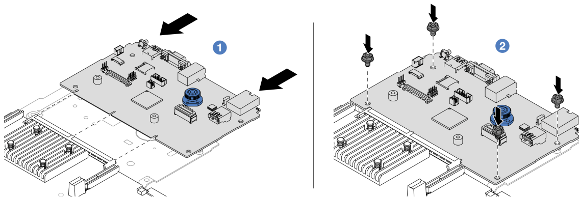
圖例 296. 將系統 I/O 板安裝在處理器板上
