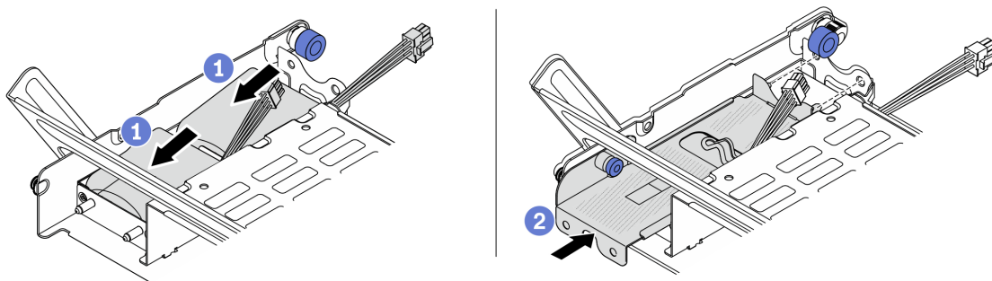
圖例 223. 將 RAID 快閃記憶體電源模組安裝在中間框架上
