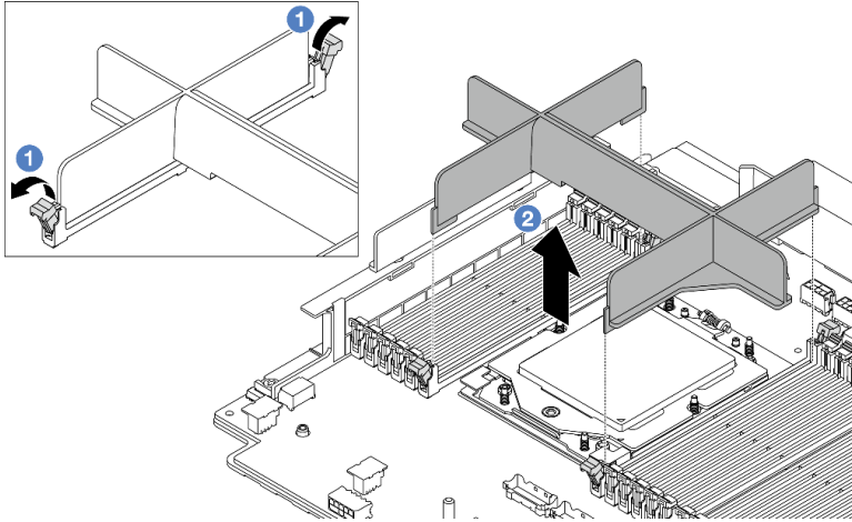
圖例 198. 卸下處理器填充板
