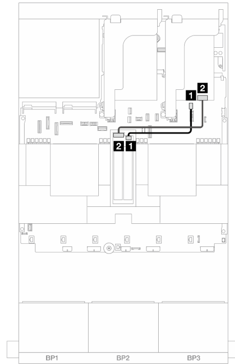
圖例 336. RAID 纜線佈線
