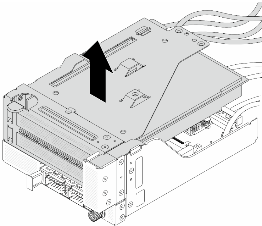
圖例 53. 抬起擴充卡 5 組件
