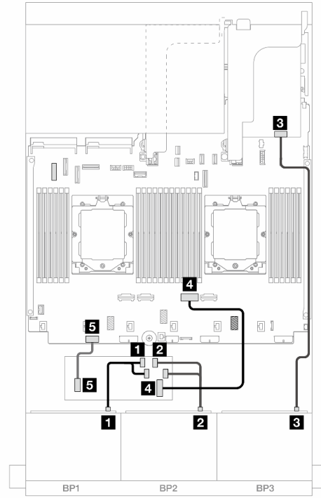
圖例 462. 安裝了一個處理器的纜線佈線
