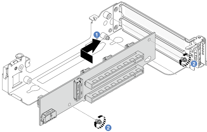
圖例 275. 將擴充卡安裝到擴充卡 3 匣
