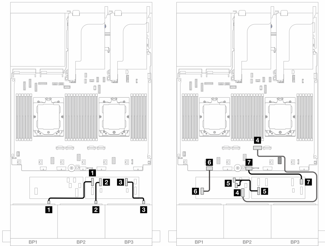
圖例 445. SAS/SATA 纜線佈線至 CFF 擴充器和 CFF 16i 配接卡
