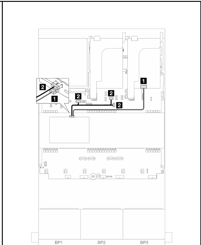
圖例 472. 中間背板纜線佈線
