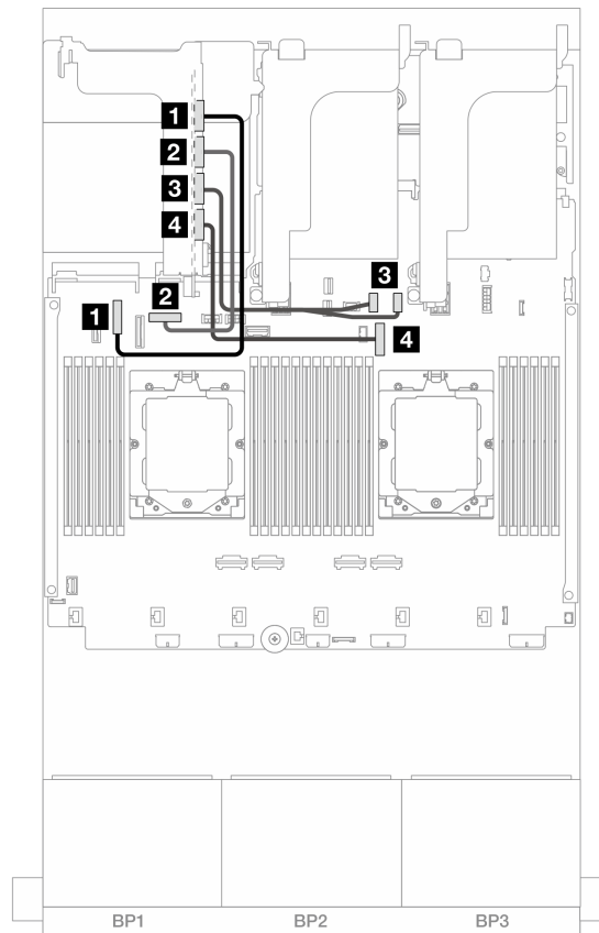
圖例 352. x16/x16 Gen 5 PCIe 擴充卡 3 的信號線連接
