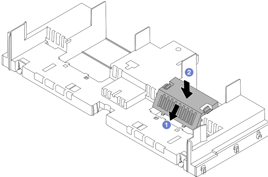
圖例 32. 安裝空氣擋板填充板
