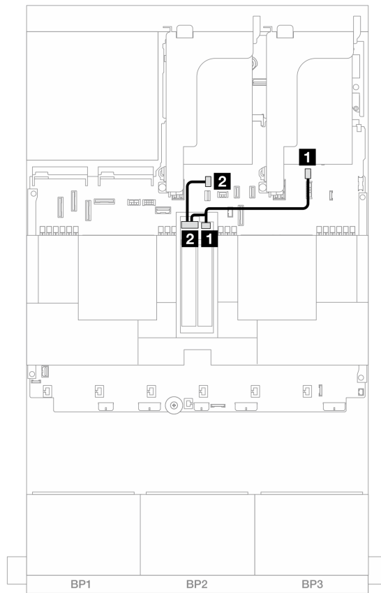
圖例 337. M.2 x1 RAID NVMe 2 機槽背板的纜線佈線
