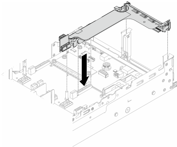
圖例 308. 安裝擴充卡組件
