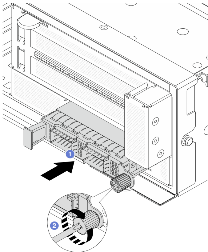
圖例 51. 安裝正面 OCP 模組
