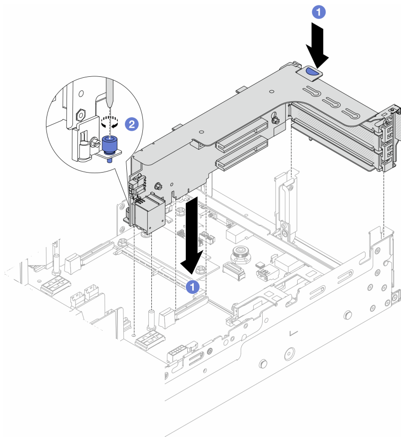
圖例 280. 安裝擴充卡 1 組件
