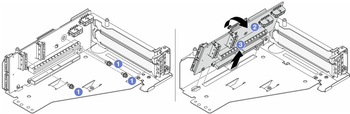
圖例 41. 從擴充卡 5 匣卸下擴充卡
