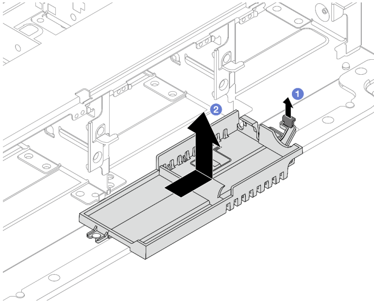
圖例 215. 卸下超級電容固定器
