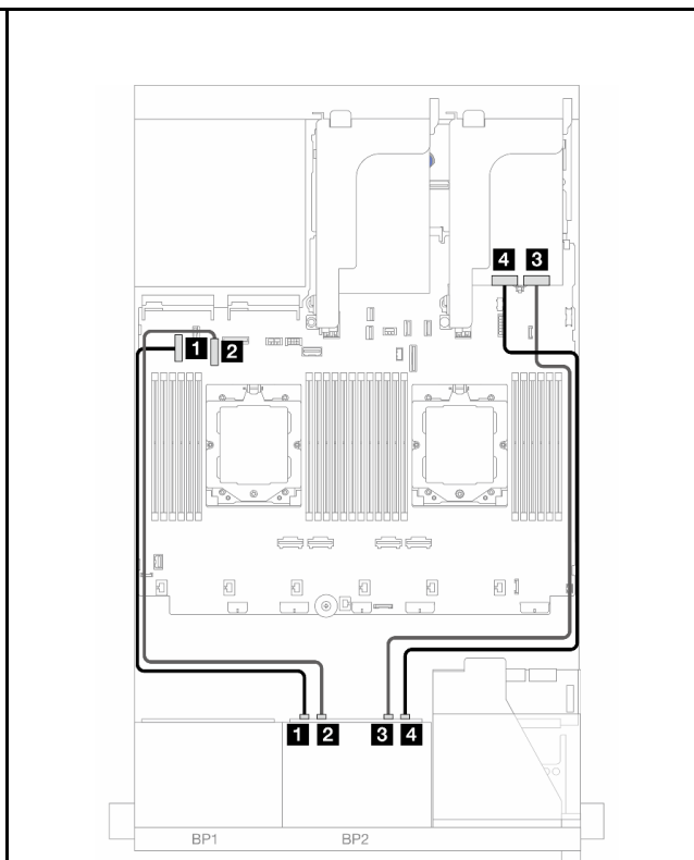
圖例 432. NVMe 纜線佈線
