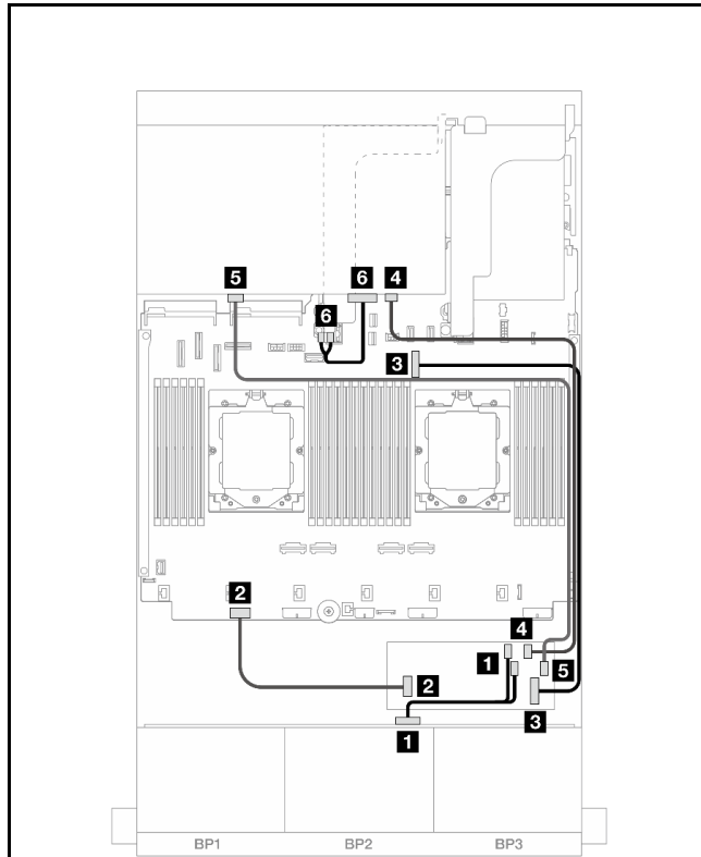
圖例 538. 安裝了兩個處理器的纜線佈線
