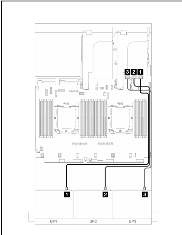
圖例 469. 前方背板纜線佈線
