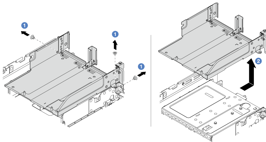
圖例 267. 卸下擴充卡匣托盤
