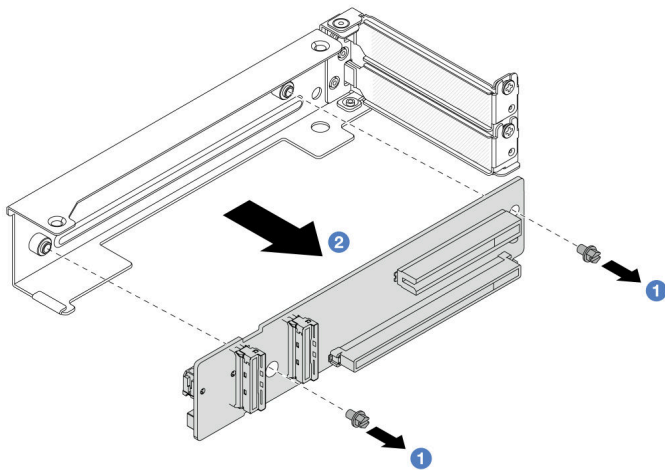
圖例 273. 從 4LP 擴充卡 3/4 匣卸下擴充卡
