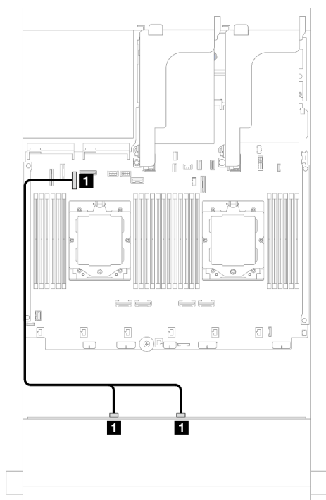
圖例 571. SAS/SATA 纜線佈線
