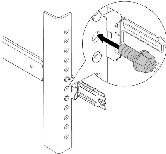
圖例 28. 將伺服器固定到機架背面
