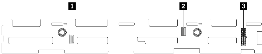
圖例 314. 8 x 3.5 吋 SAS/SATA 背板接頭
