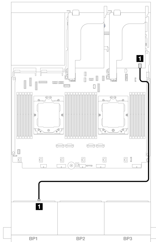
圖例 365. SAS/SATA 纜線佈線至 8i/16i RAID/HBA 配接卡
