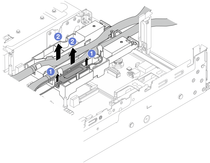
圖例 103. 拔開水管和模組
