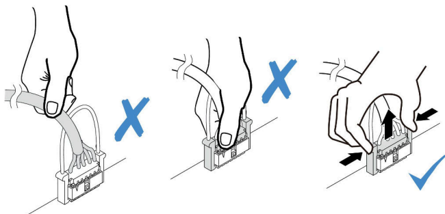
圖例 302. 從系統 I/O 板上拔掉纜線
