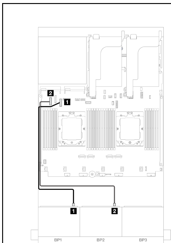
圖例 388. 安裝了兩個處理器的纜線佈線
