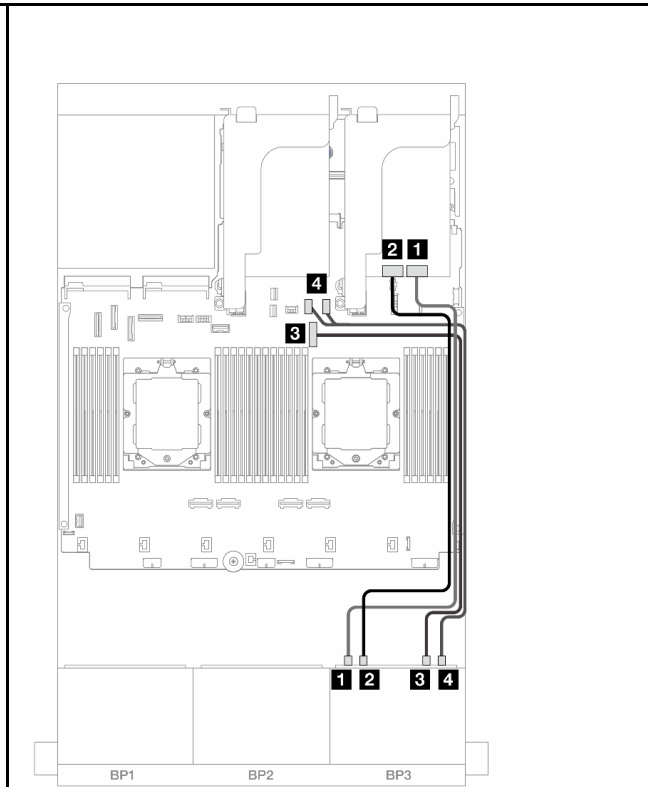
圖例 525. NVMe 纜線佈線
