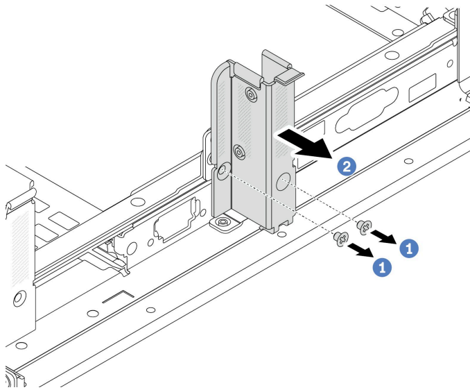
圖例 227. 卸下 B1 後壁托架 (中)
