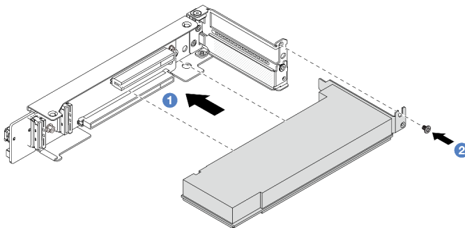
圖例 279. 將 PCIe 配接卡安裝到 4LP 擴充卡 3/4 組件
