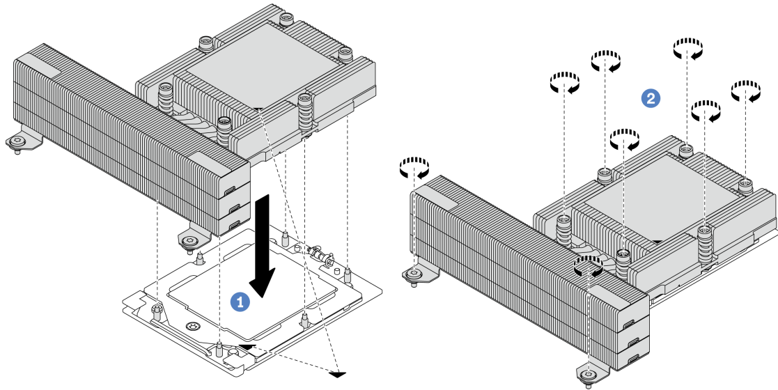
圖例 202. 安裝效能散熱槽
