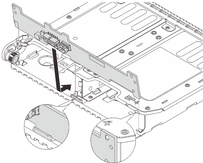
圖例 253. 安裝 2 x 3.5 吋後方硬碟背板
