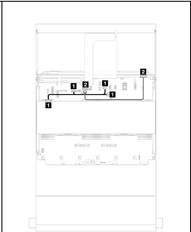
圖例 566. 後方背板電源線佈線
