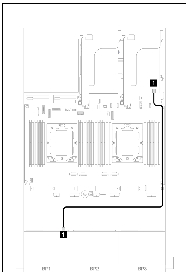
圖例 499. SAS/SATA 纜線佈線
