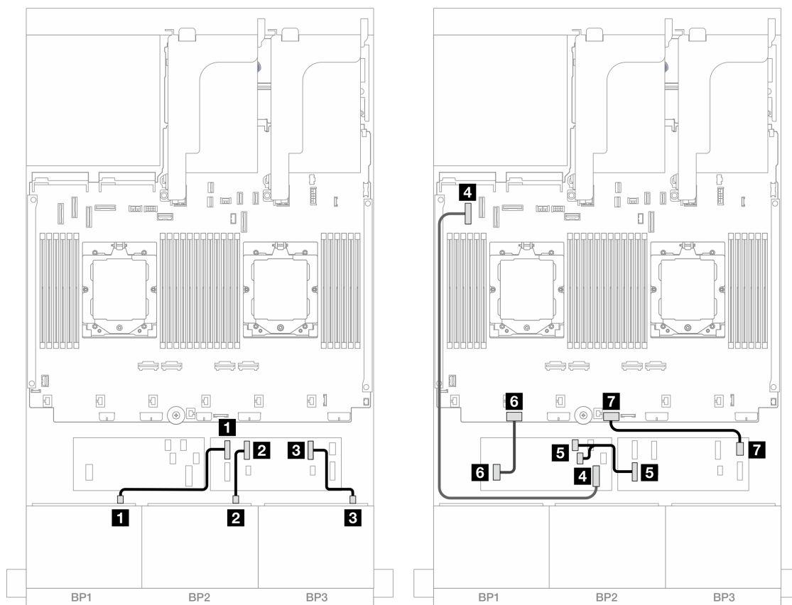
圖例 486. SAS/SATA 纜線佈線至 CFF 擴充器和 CFF 16i 配接卡
