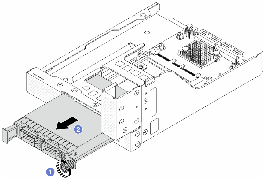
圖例 42. 卸下 OCP 模組
