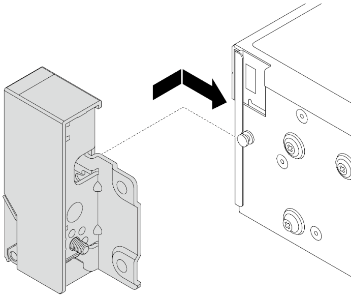
圖例 207. 安裝機架門鎖
