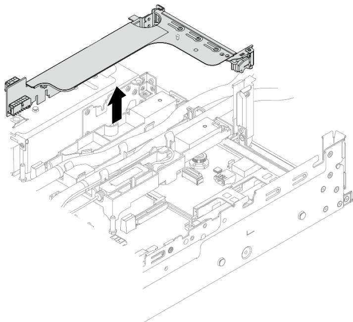
圖例 101. 卸下 1FH 擴充卡匣
