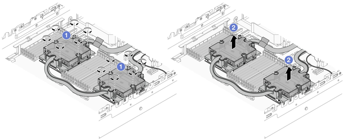
圖例 104. 卸下 DWCM
