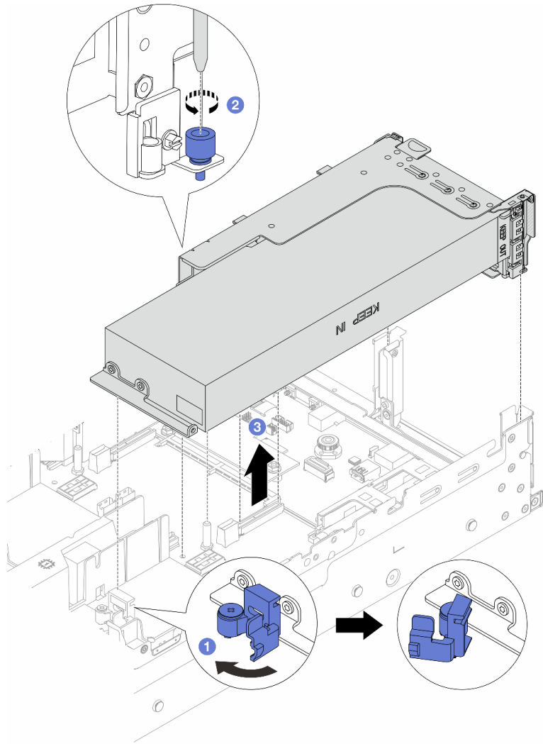
圖例 88. 卸下配備 GPU 配接卡的擴充卡 1 組件
