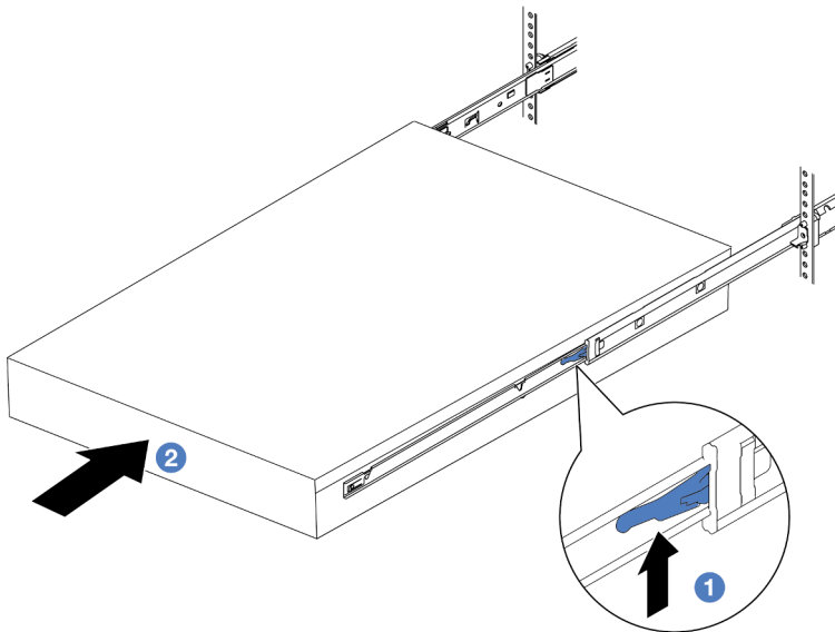
圖例 27. 將伺服器安裝到機架中
