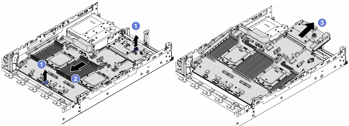
圖例 292. 卸下主機板組件
