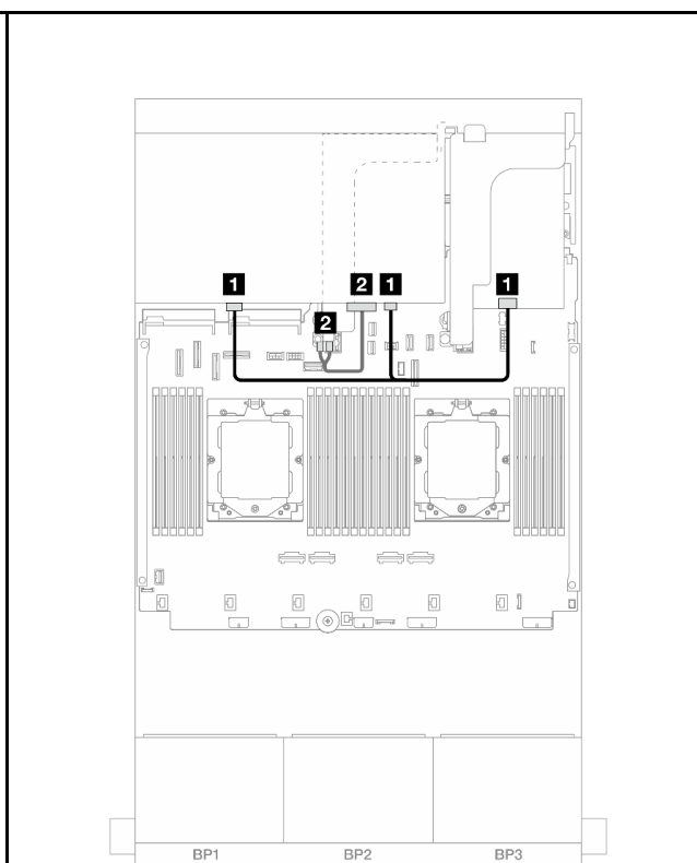
圖例 460. 後方背板纜線佈線
