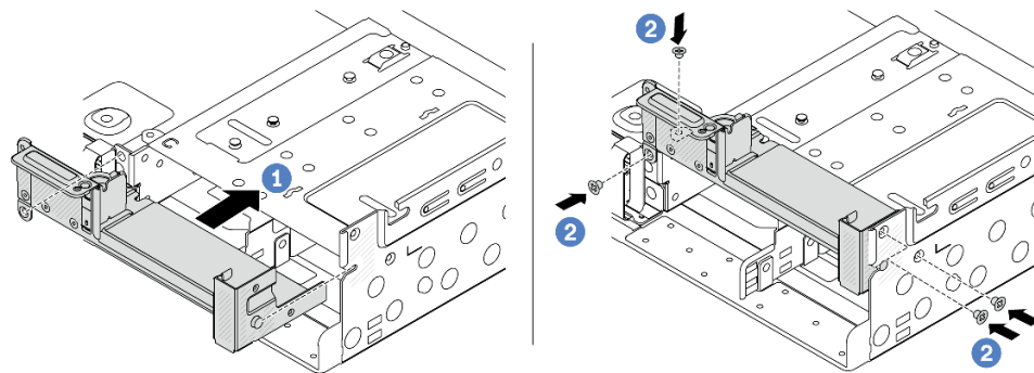
圖例 231. 安裝 C1 後壁托架 (右)
