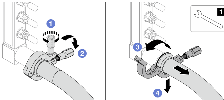
圖例 167. 將歧管與軟管套件分離
