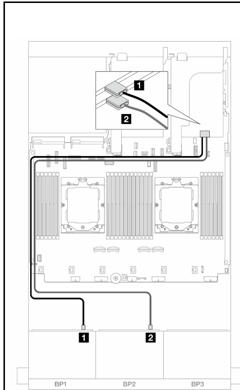
圖例 524. SAS/SATA 纜線佈線
