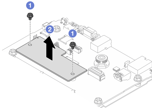
圖例 290. 卸下韌體和 RoT 安全模組
