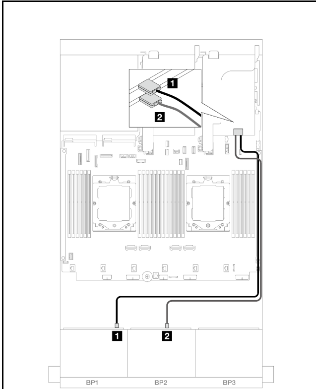
圖例 418. SAS/SATA 纜線佈線
