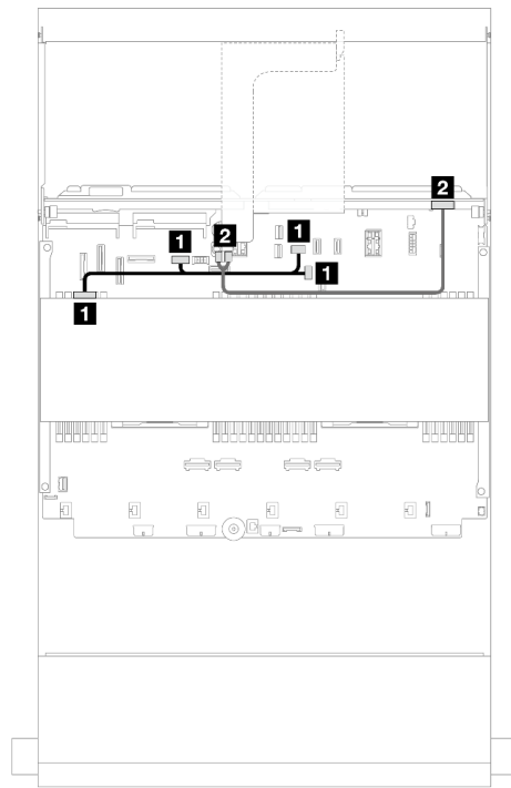
圖例 586. 中間/後方背板電源線佈線
