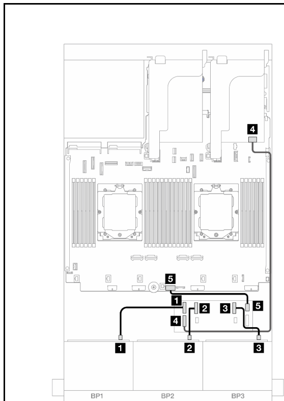
圖例 442. 前方背板纜線佈線
