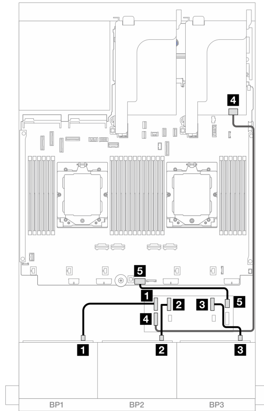
圖例 479. SAS/SATA 纜線佈線至 CFF 擴充器和 8i/16i 配接卡
