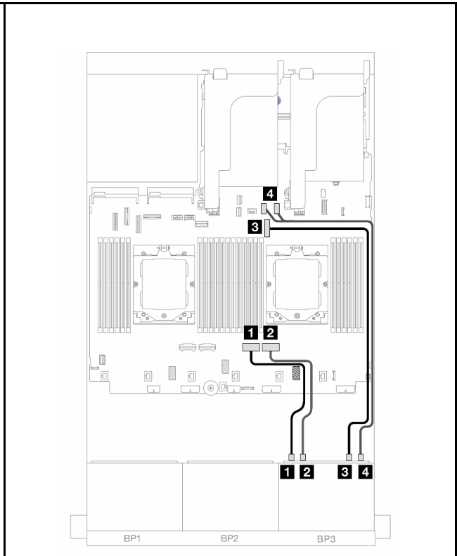
圖例 509. NVMe 纜線佈線
