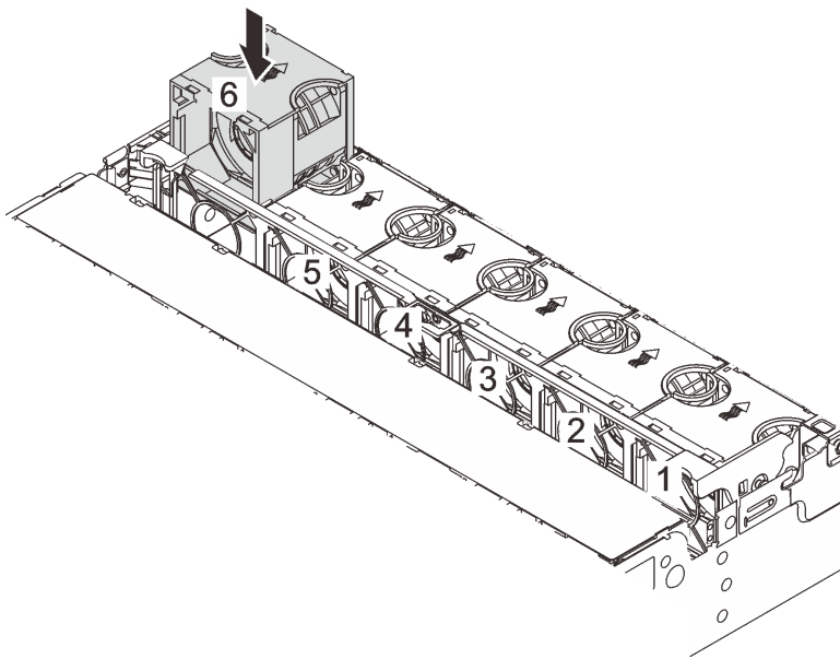
圖例 299. 安裝系統風扇
