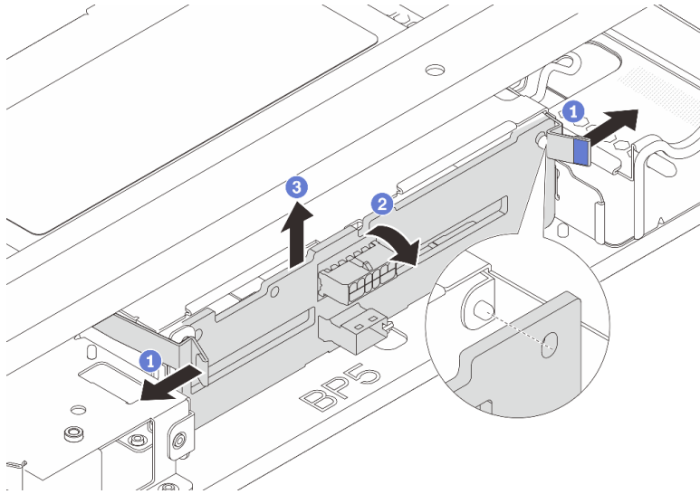
圖例 184. 卸下中間 2.5 吋硬碟背板
