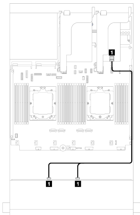
圖例 575. SAS/SATA 纜線佈線
