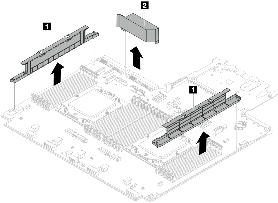
圖例 601. 從處理器板上卸下元件
