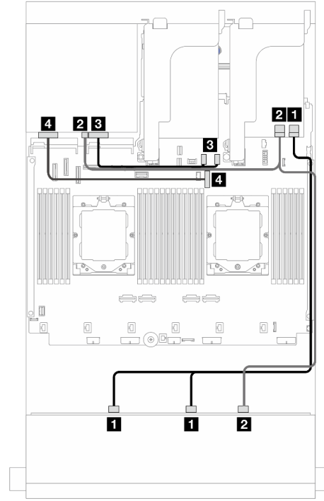
圖例 556. 安裝了一個處理器的纜線佈線
