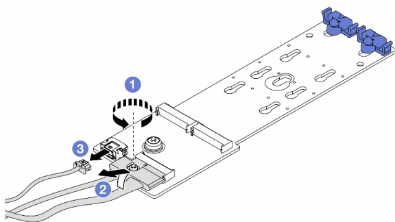
圖例 118. 從 M.2 x4 非 RAID SATA/NVMe 2 機槽背板拔掉纜線
