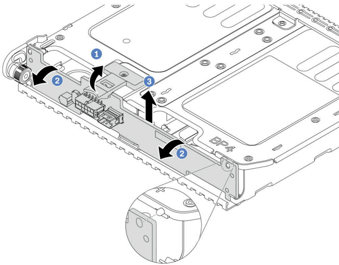
圖例 252. 卸下 2 x 3.5 吋後方硬碟背板
