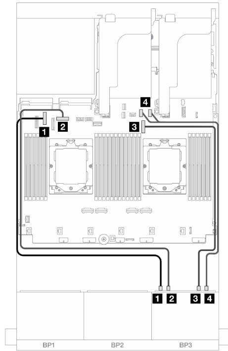
圖例 507. NVMe 纜線佈線
