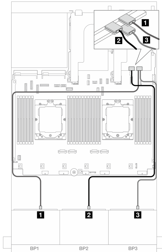
圖例 490. SAS/SATA 纜線佈線至 8i/16i 三模式配接卡
