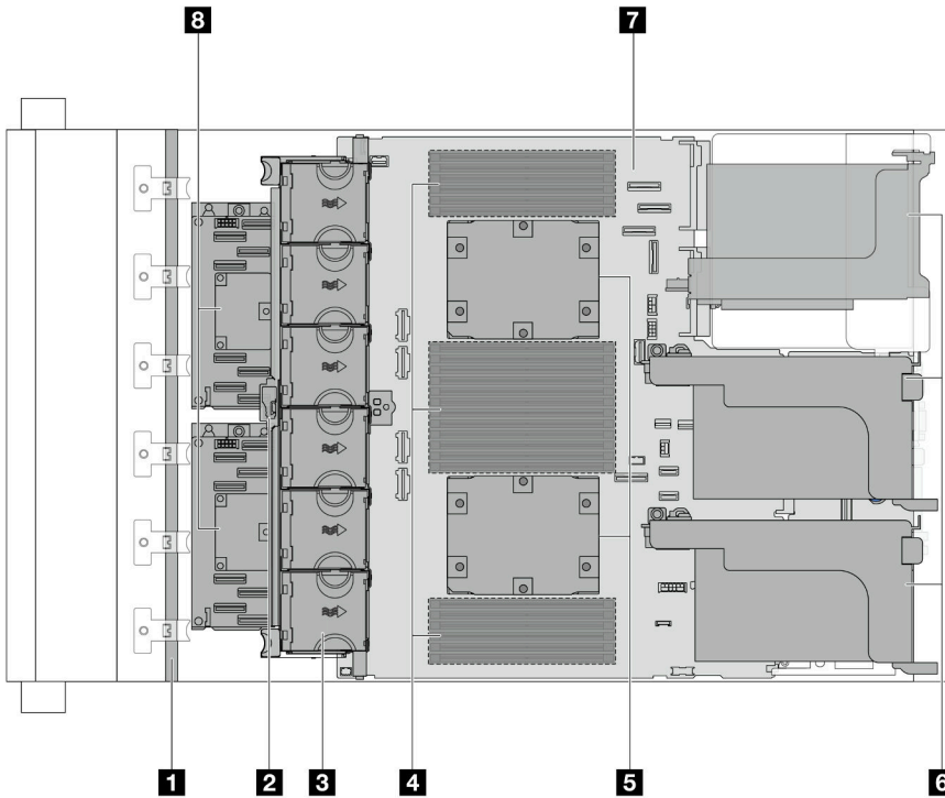
圖例 9. 配備標準散熱槽的俯視圖
