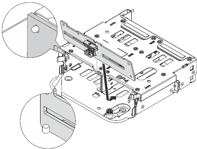
圖例 245. 安裝 4 x 2.5 吋後方硬碟背板
