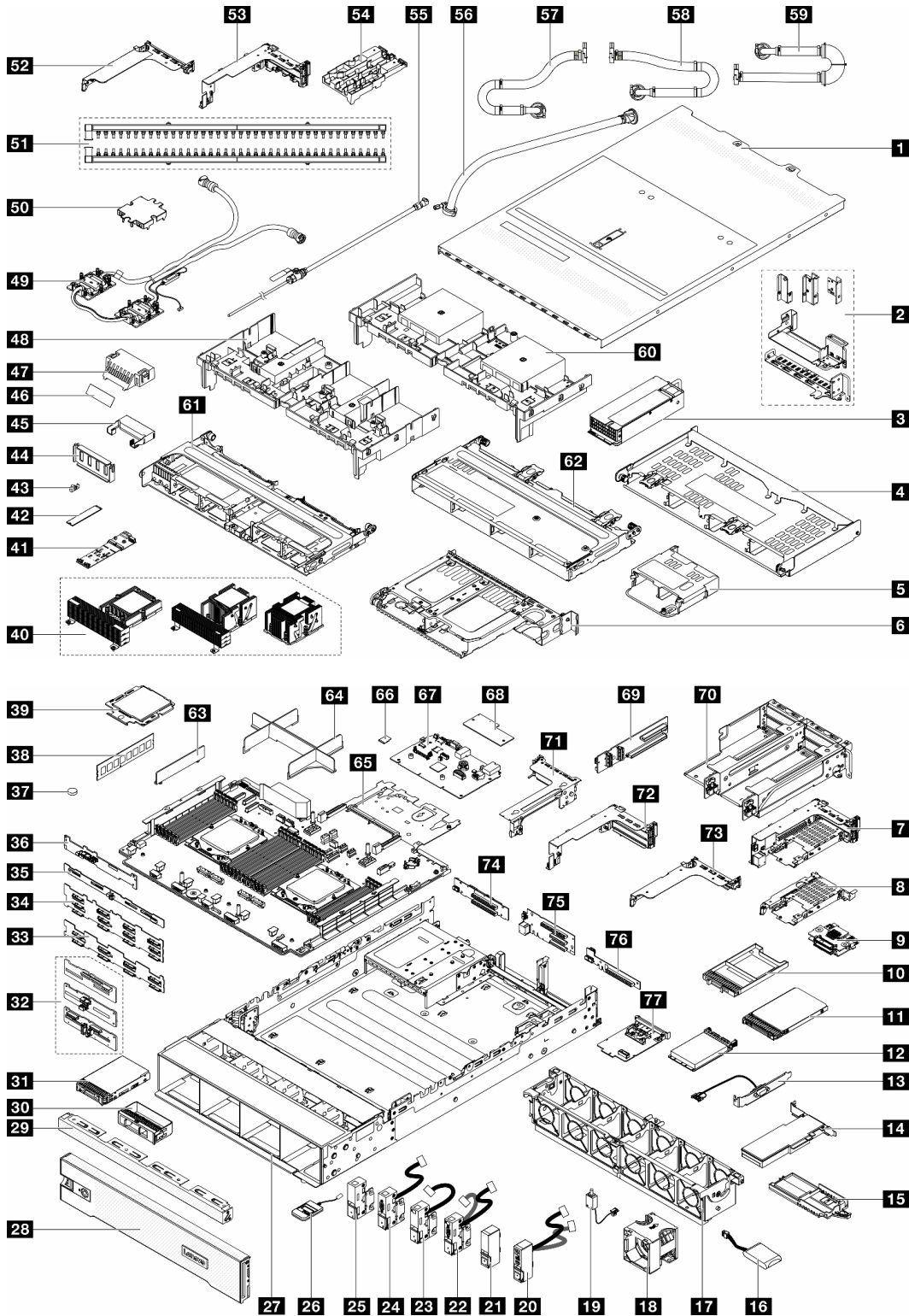
圖例 15. 伺服器元件 (3.5 吋機槽機箱)
