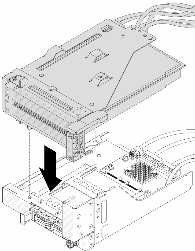
圖例 68. 將擴充卡 5 組件安裝到正面 OCP 組件上
