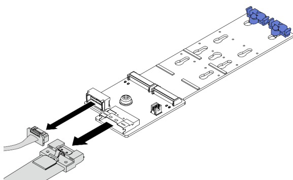
圖例 118. 從 M.2 x4 非 RAID SATA/NVMe 2 機槽背板拔掉纜線
