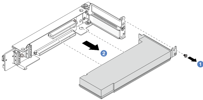
圖例 270. 從 4LP 擴充卡 3/4 組件卸下 PCIe 配接卡
