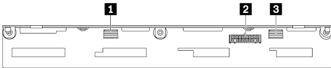
圖例 322. 8x2.5 吋 SAS/SATA 背板接頭
