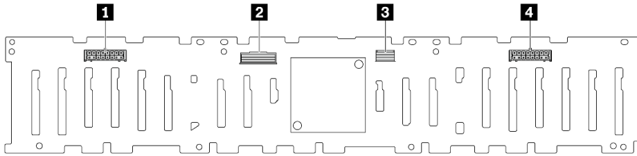
圖例 313. 24 x 2.5 吋 SAS/SATA 擴充器背板上的接頭
