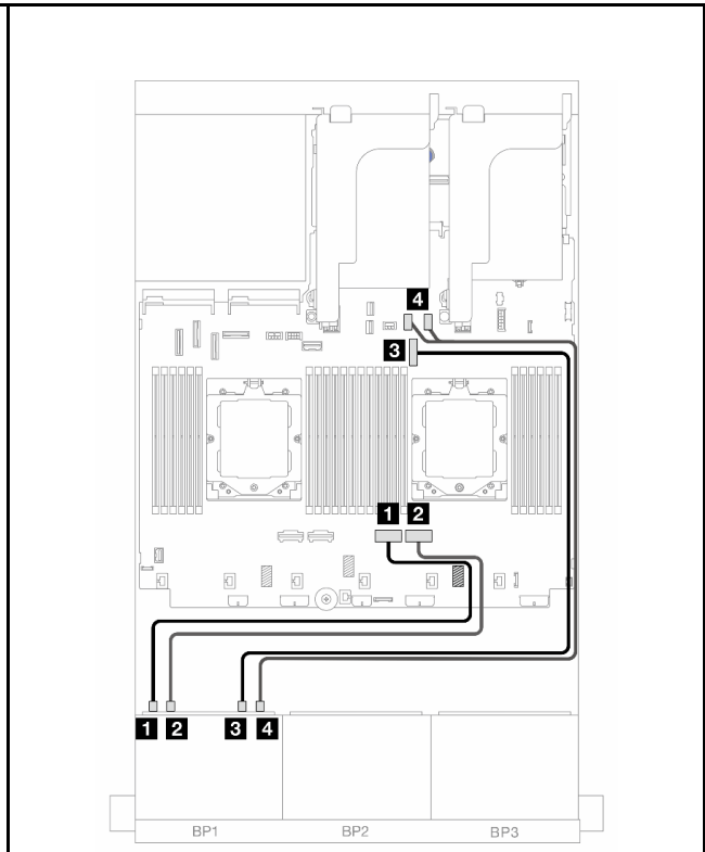
圖例 385. 安裝了一個處理器的纜線佈線
