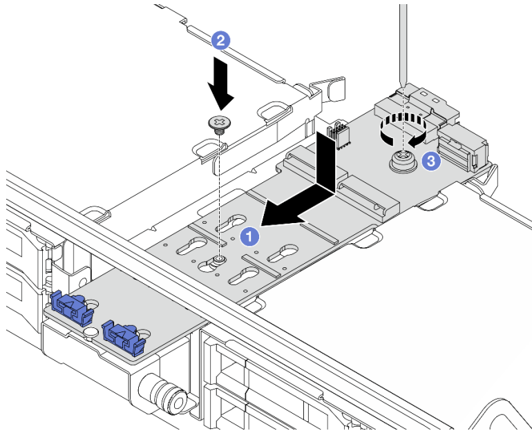
圖例 125. 將 M.2 背板安裝在中間框架上
