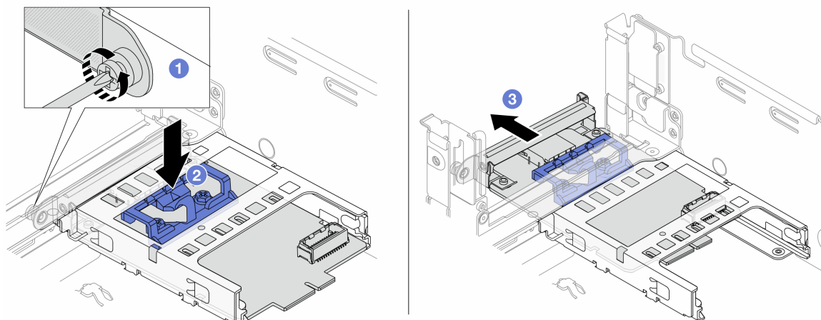
圖例 130. 卸下管理 NIC 配接卡
