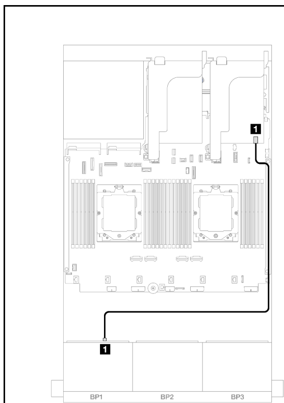
圖例 380. SAS/SATA 纜線佈線
