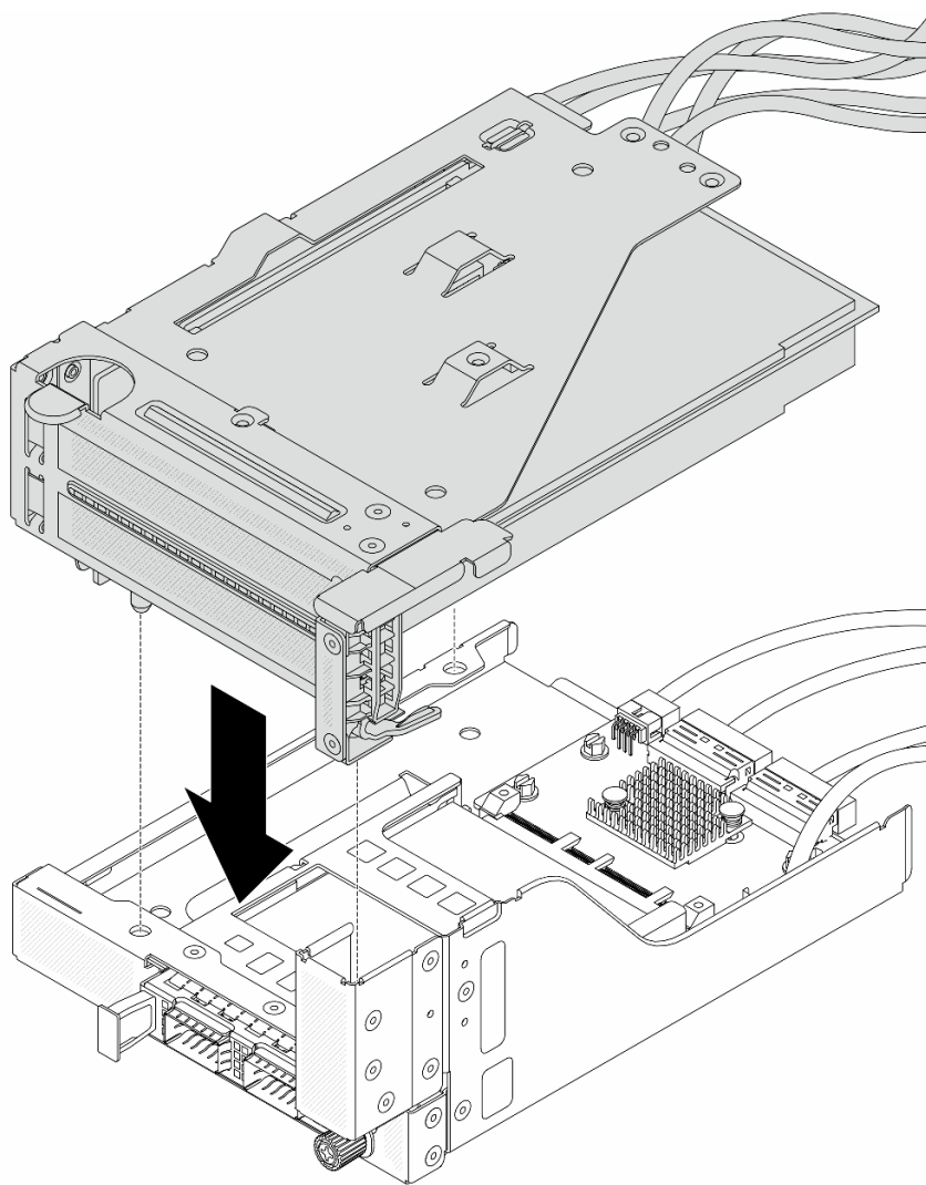
圖例 58. 將擴充卡 5 組件安裝到正面 OCP 組件上
