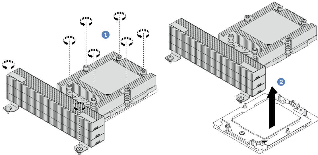
圖例 195. 卸下效能散熱槽
