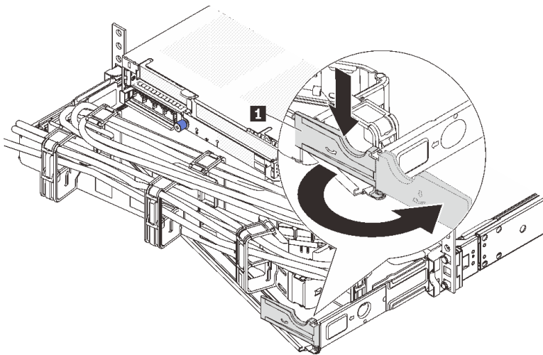
圖例 189. 調整 CMA
