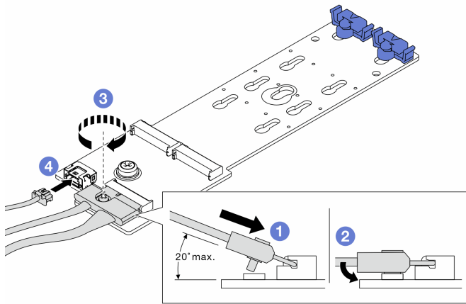
圖例 128. 將 M.2 纜線連接至 M.2 x1 RAID NVMe 2 機槽背板
