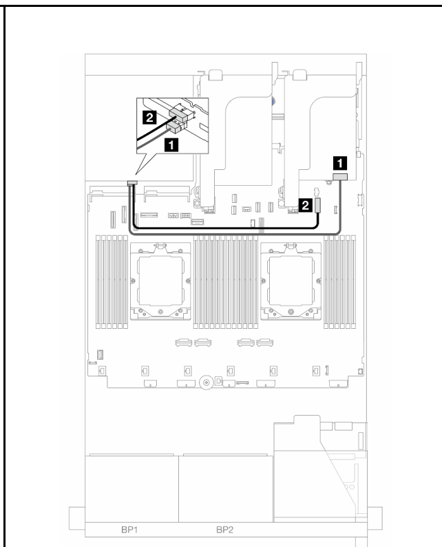
圖例 401. 後方背板纜線佈線
