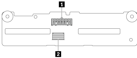
圖例 318. 4 x 2.5 吋 SAS/SATA 背板接頭
