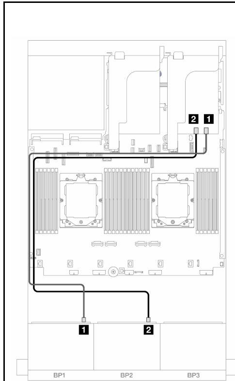
圖例 528. SAS/SATA 纜線佈線
