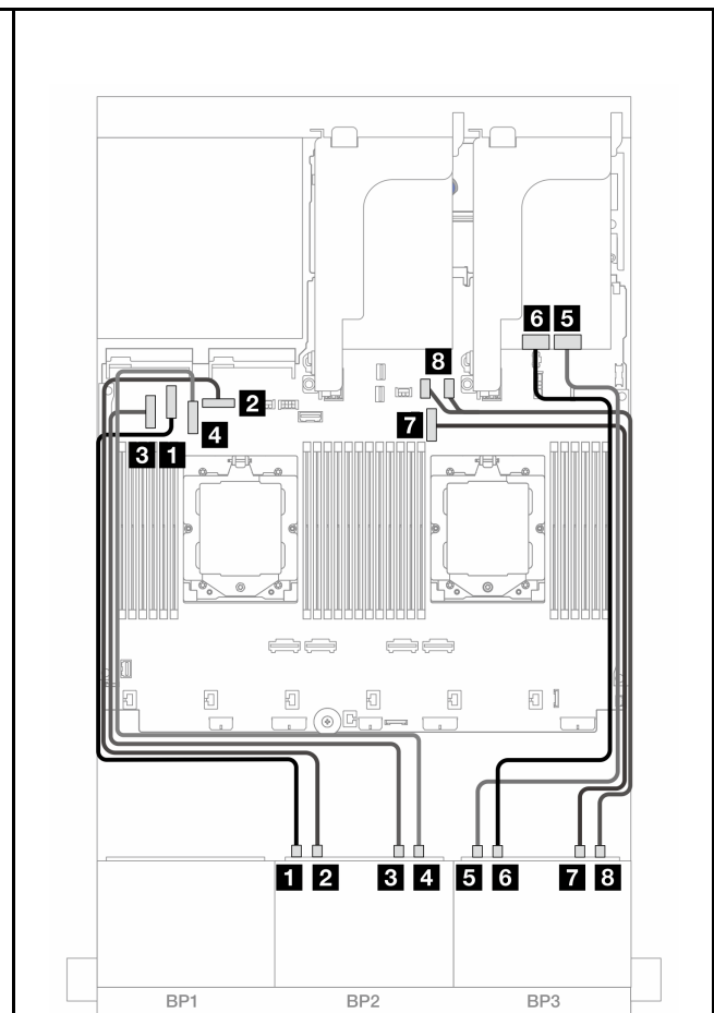
圖例 502. NVMe 纜線佈線
