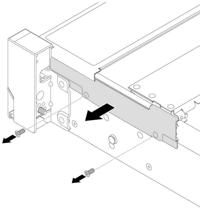
圖例 204. 卸下纜線固定夾
