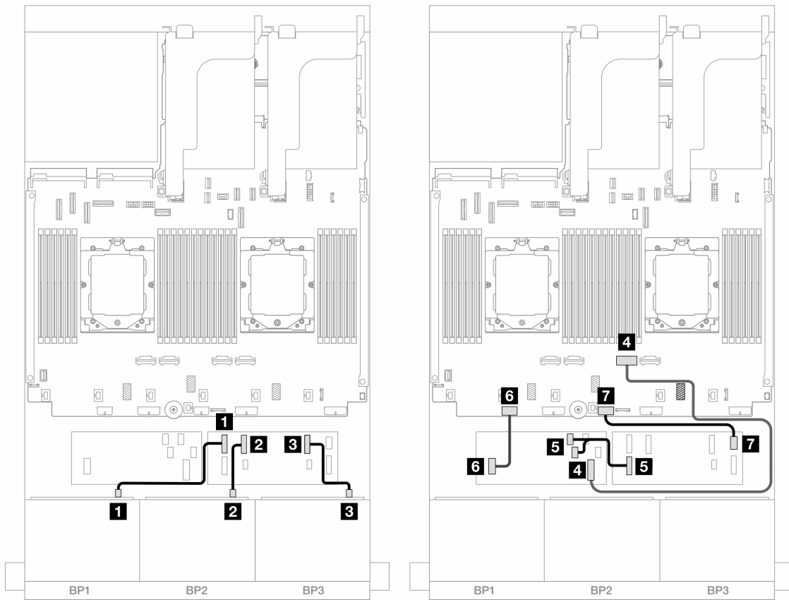
圖例 454. SAS/SATA 纜線佈線至 CFF 擴充器和 CFF 16i 配接卡
