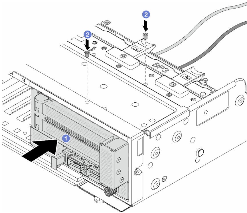
圖例 59. 安裝前配接器組件
