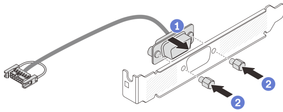
圖例 306. 組裝序列埠模組
