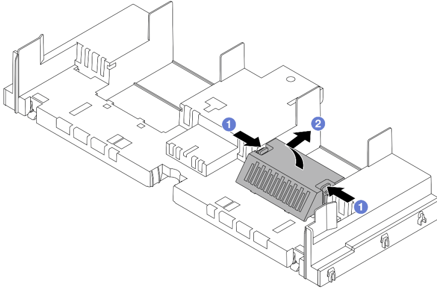
圖例 31. 卸下空氣擋板填充板
