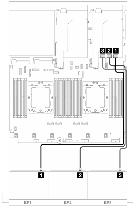
圖例 457. 前方背板纜線佈線
