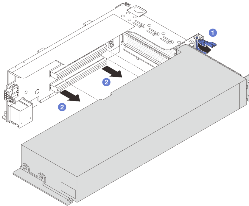
圖例 90. 卸下 GPU 配接卡
