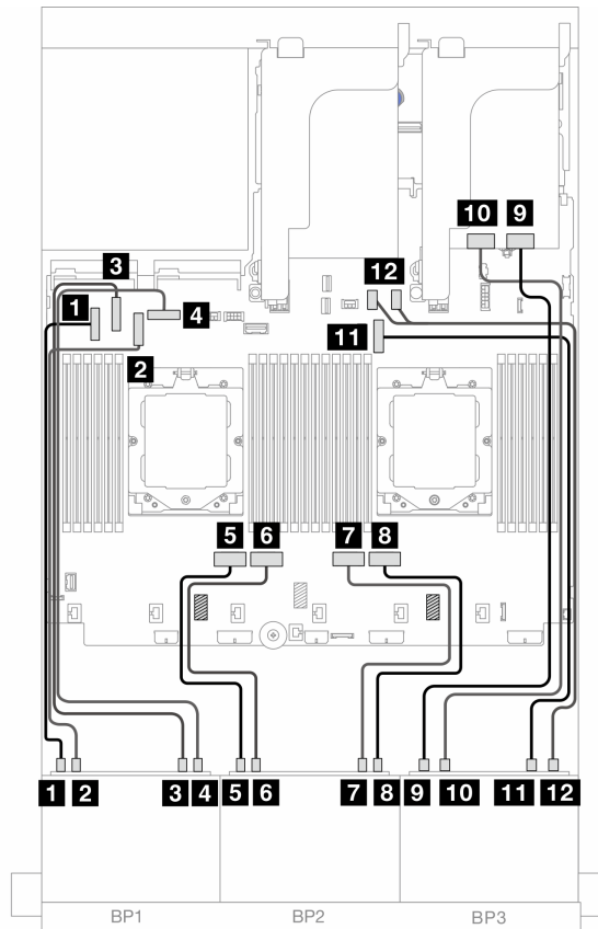
圖例 496. NVMe 纜線佈線至機載接頭和重定時器卡
