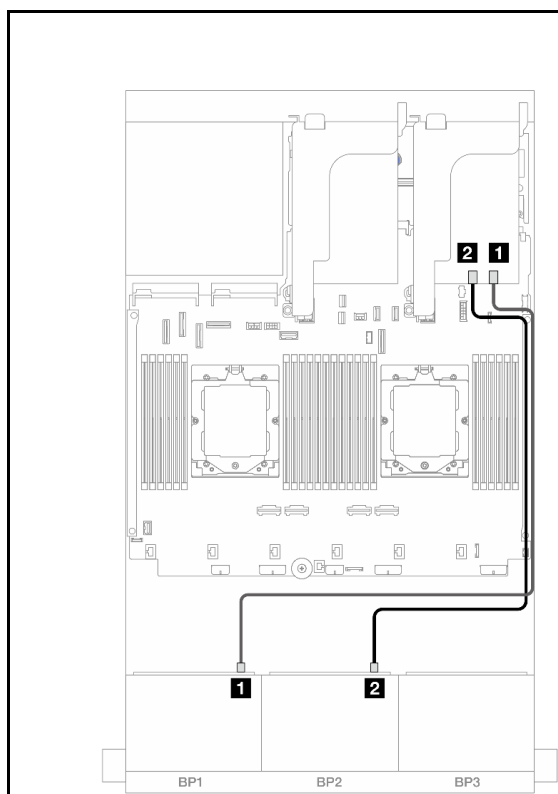
圖例 395. 前方背板纜線佈線
