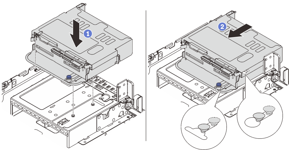
圖例 246. 安裝 4 x 2.5 吋背面框架
