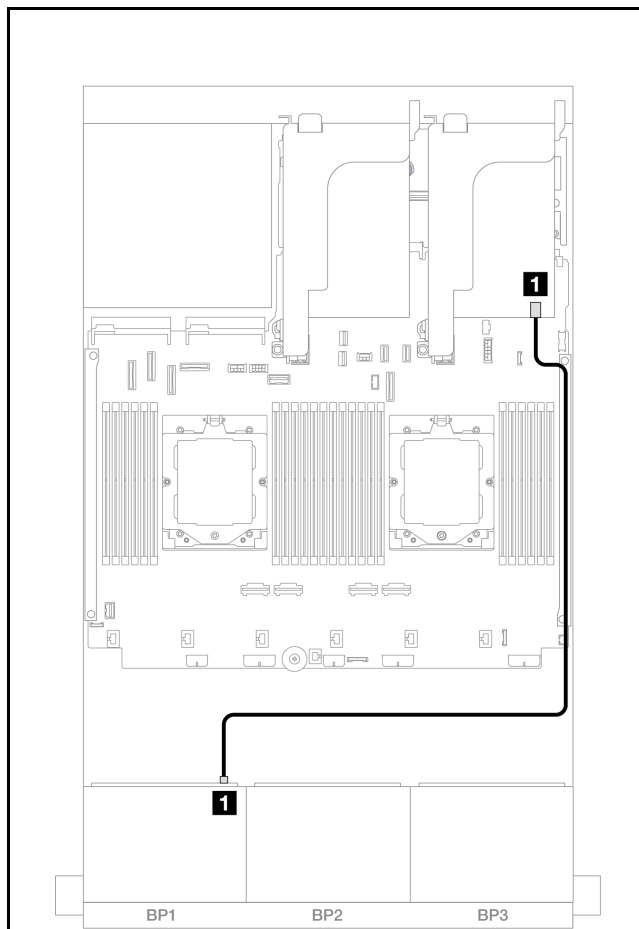
圖例 501. SAS/SATA 纜線佈線
