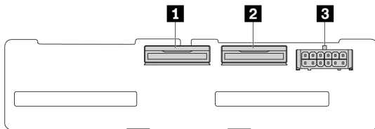
圖例 319. 4 x 2.5 吋 NVMe 背板接頭
