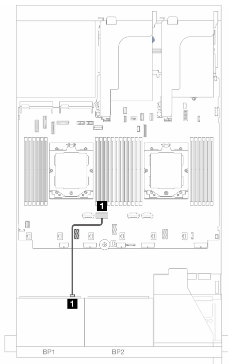
圖例 381. NVMe 纜線佈線
