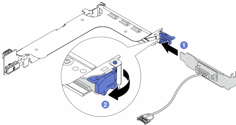
圖例 307. 安裝序列埠模組
