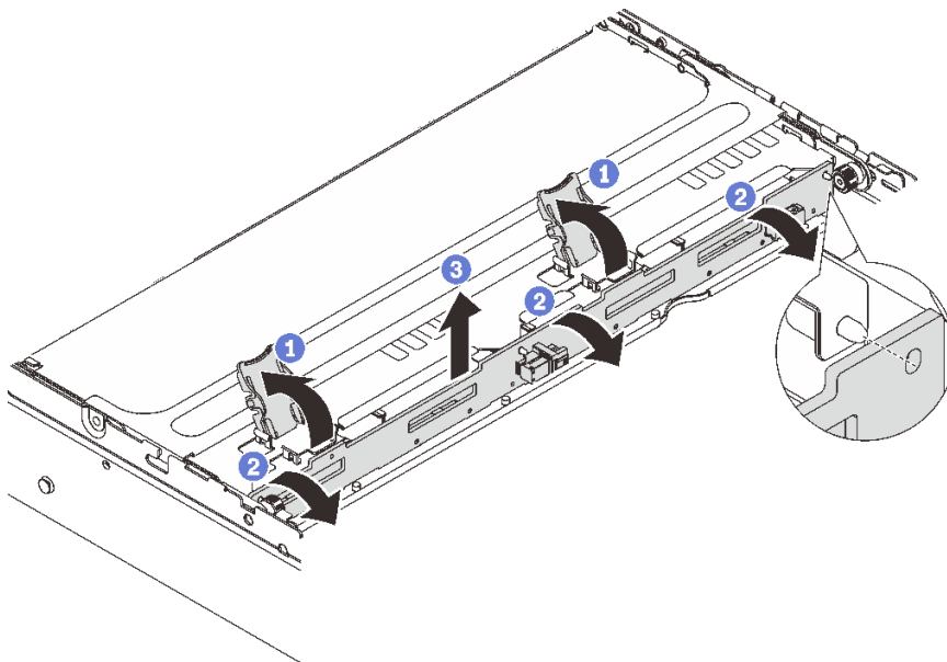
圖例 185. 卸下中間 3.5 吋硬碟背板
