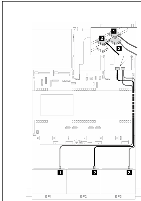
圖例 471. 前方背板纜線佈線
