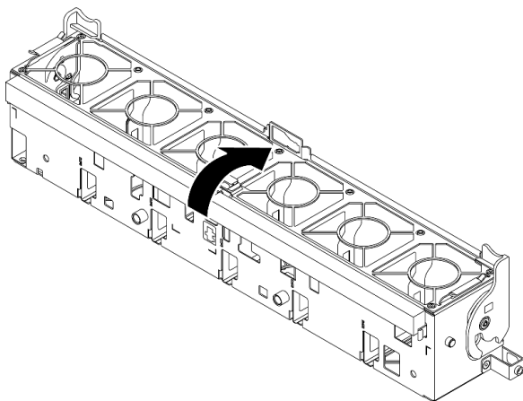
圖例 98. 旋轉風扇機盒
