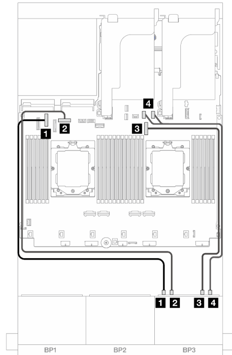
圖例 521. NVMe 纜線佈線
