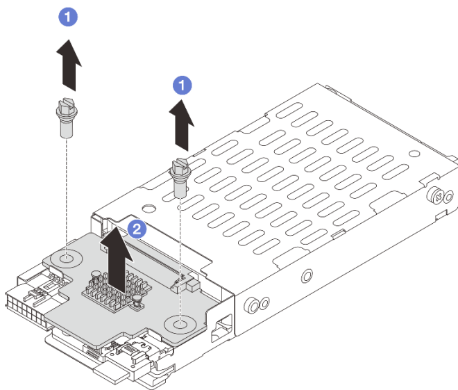
圖例 235. 卸下 7 公釐硬碟背板 (頂端)
