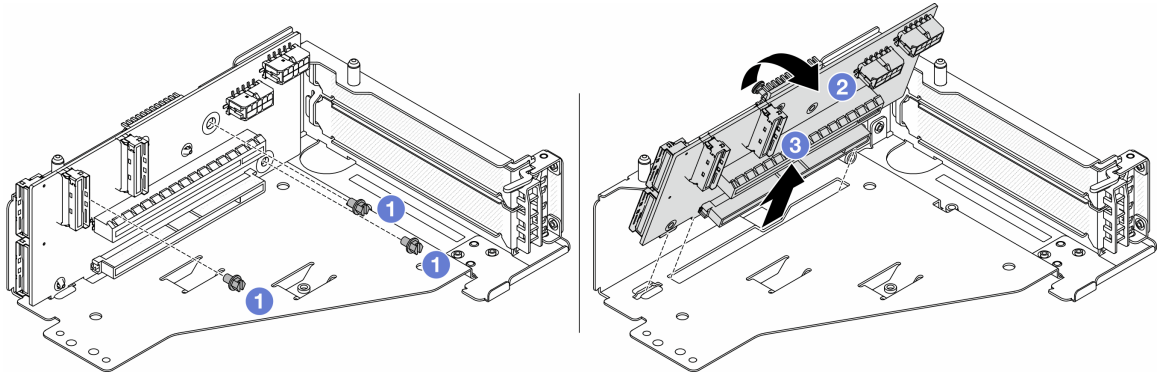
圖例 65. 從擴充卡 5 匣卸下擴充卡
