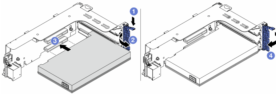
圖例 277. 將 PCIe 配接卡安裝到擴充卡 1 或 2 組件
