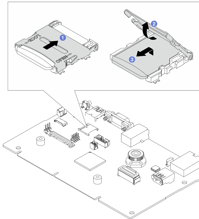
圖例 294. 卸下 MicroSD 卡
