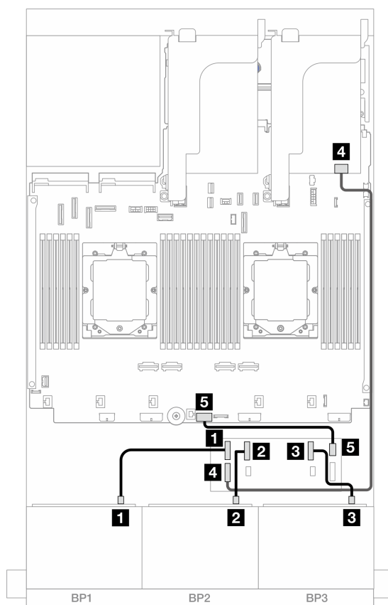
圖例 484. SAS/SATA 纜線佈線至 CFF 擴充器和 16i 配接卡
