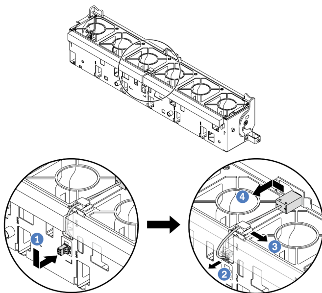
圖例 99. 卸下入侵開關
