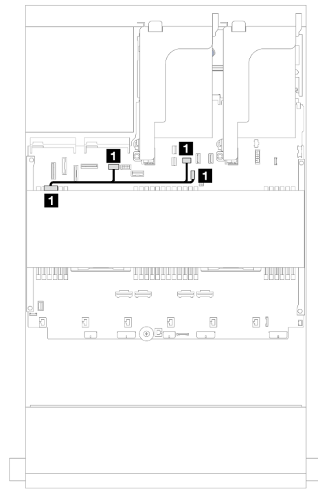
圖例 559. 中間背板電源線佈線
