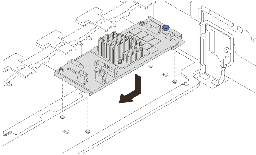
圖例 97. 安裝內部 CFF 配接卡
