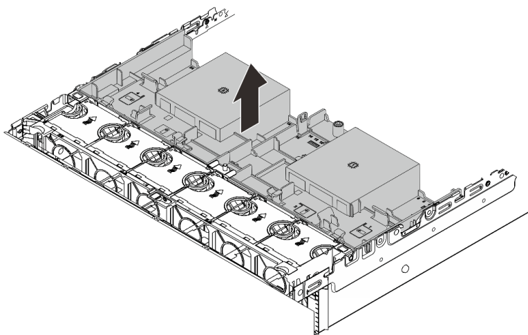
圖例 30. 卸下空氣擋板
