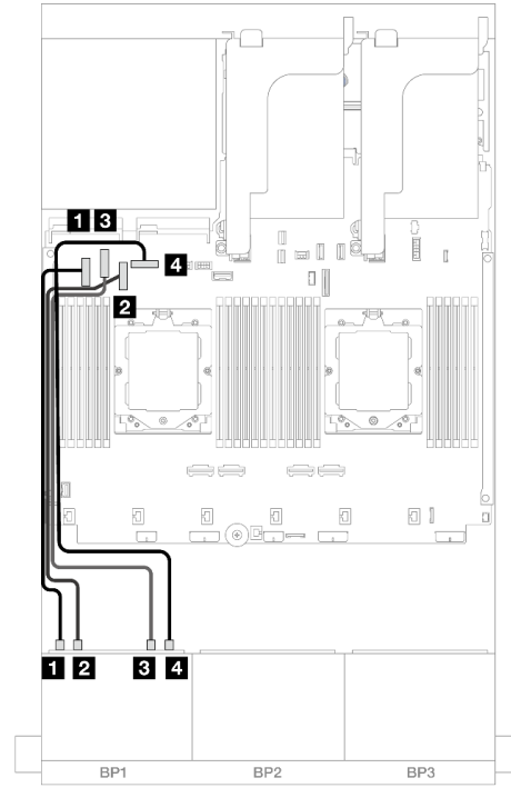
圖例 369. NVMe 纜線佈線
