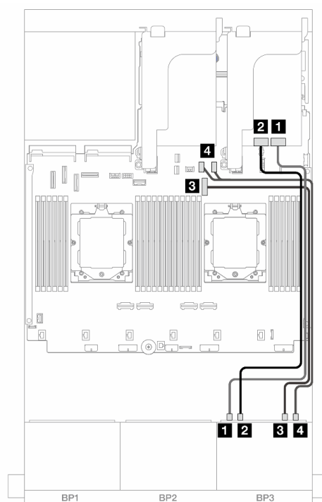
圖例 531. NVMe 纜線佈線
