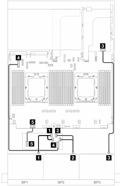
圖例 461. 安裝了兩個處理器的纜線佈線
