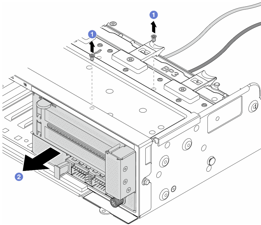
圖例 62. 卸下前配接器組件
