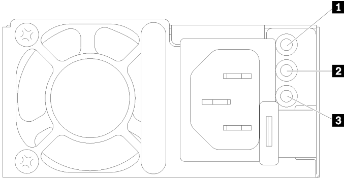
圖例 593. 電源供應器 LED
