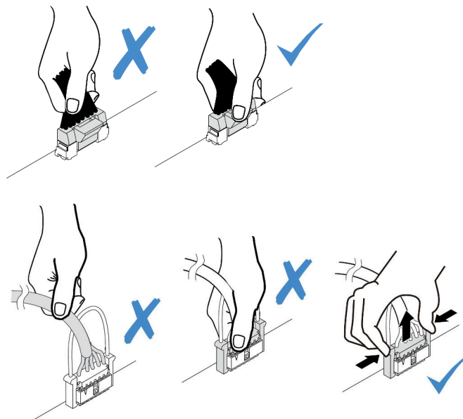
圖例 203. 從主機板組件拔掉纜線
