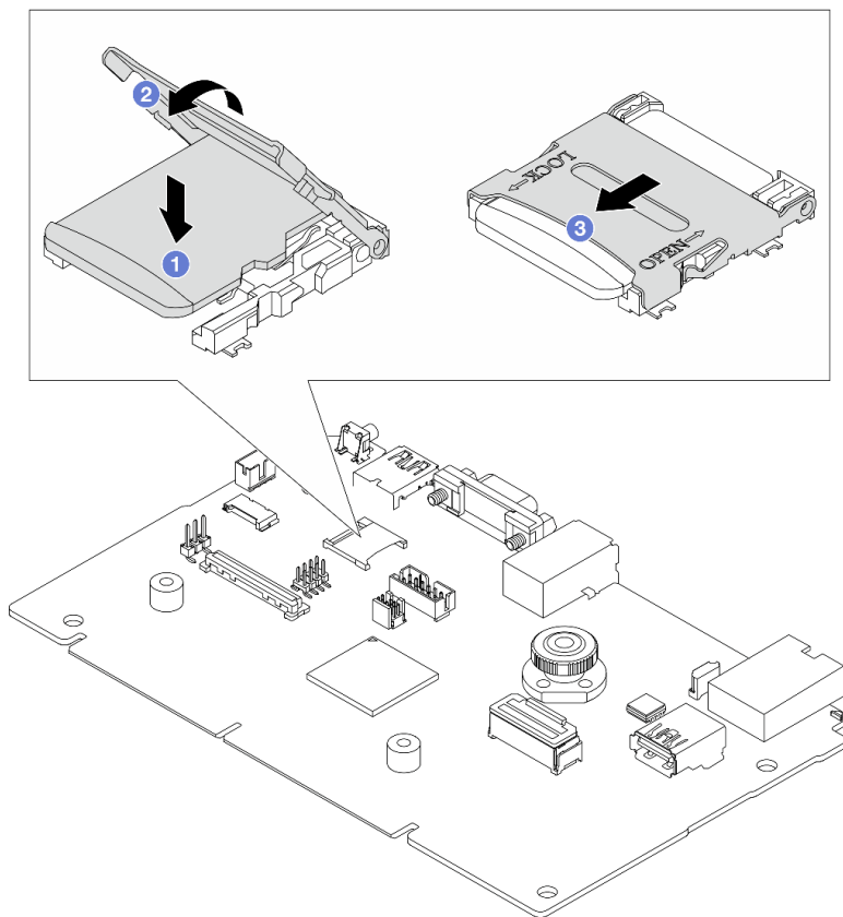
圖例 182. 安裝 MicroSD 卡
