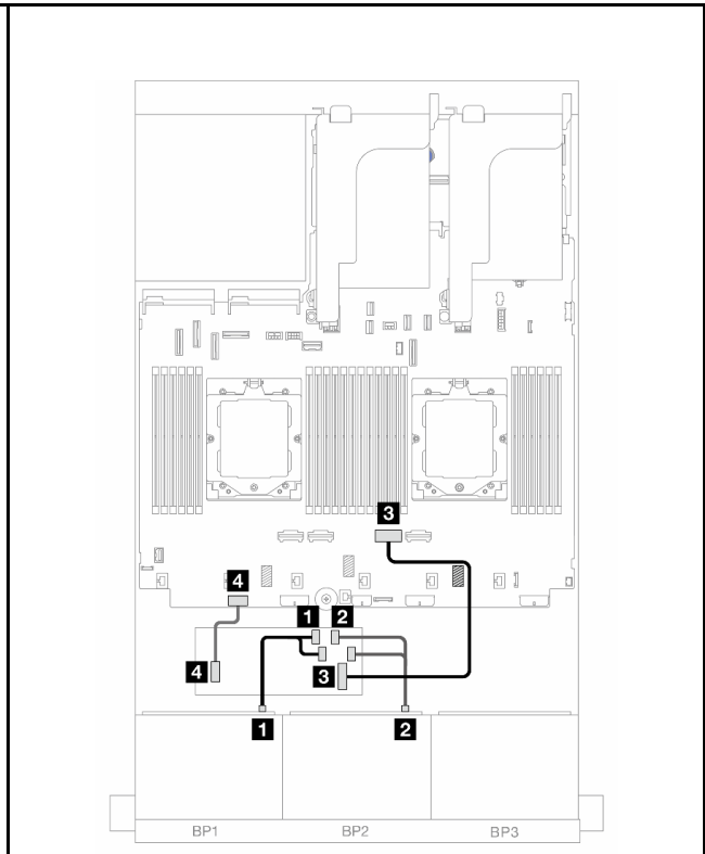
圖例 392. 安裝了一個處理器的纜線佈線
