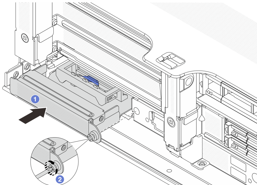
圖例 61. 安裝背面 OCP 轉插卡
