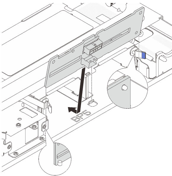
圖例 186. 安裝中間 2.5 吋硬碟背板
