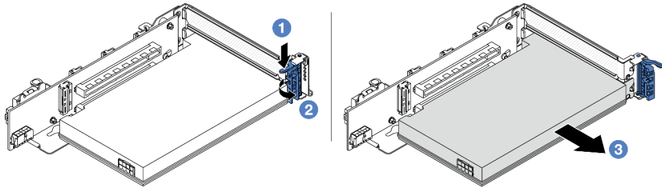
圖例 269. 從擴充卡 3 組件卸下 PCIe 配接卡
