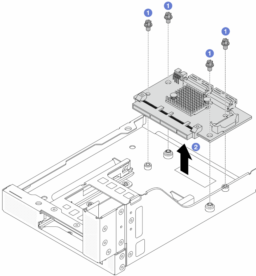
圖例 55. 卸下正面 OCP 轉插卡
