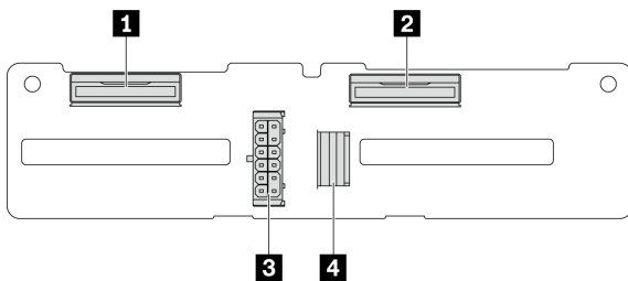
圖例 323. 4 x 2.5 吋 AnyBay 背板接頭
