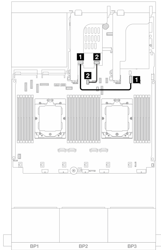
圖例 327. 7 公釐 RAID NVMe 2 機槽背板的纜線佈線
