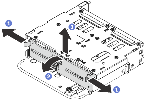
圖例 244. 卸下 4 x 2.5 吋後方硬碟背板
