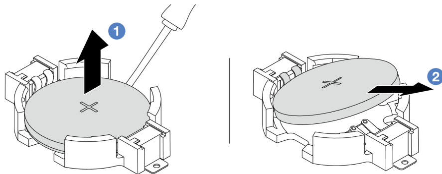
圖例 36. 取出 CMOS 電池
