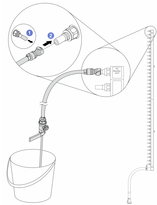
圖例 165. 在回流側安裝洩放套件
