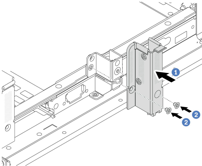
圖例 230. 安裝 B1 後壁托架 (中)
