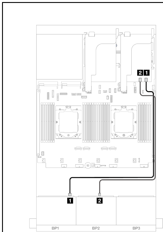
圖例 420. SAS/SATA 纜線佈線
