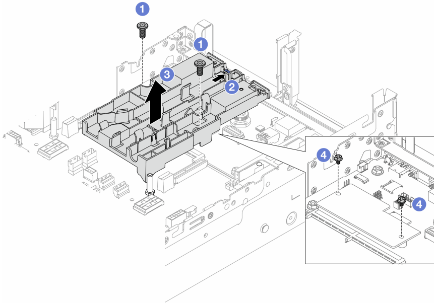
圖例 105. 卸下水管固定器
