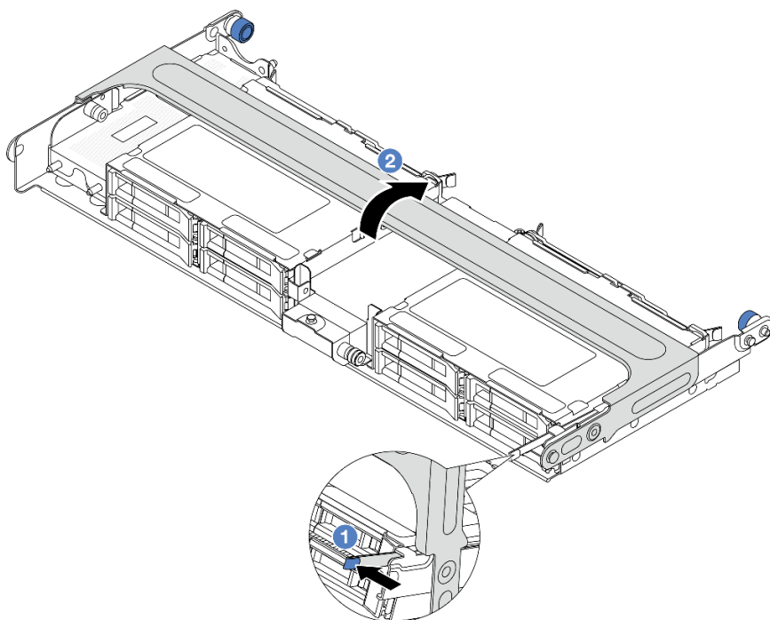
圖例 224. 關上中間框架的把手
