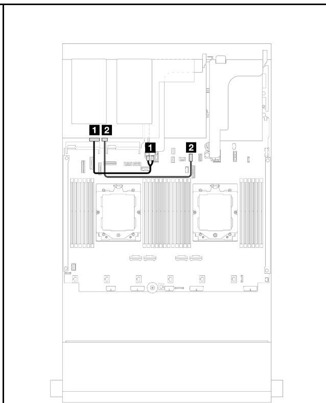
圖例 550. 安裝了一個處理器的纜線佈線
