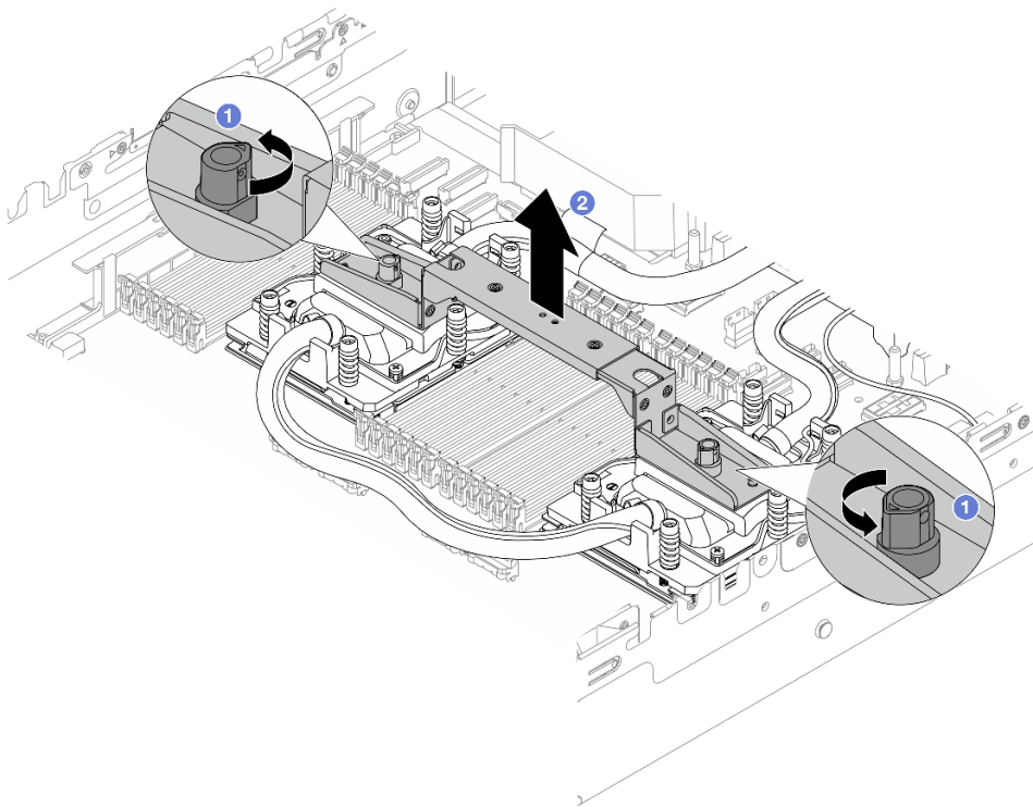
圖例 108. 卸下模組把手
