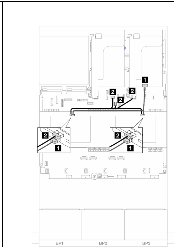
圖例 476. 中間背板纜線佈線
