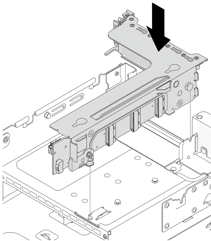
圖例 281. 安裝擴充卡 3 組件
