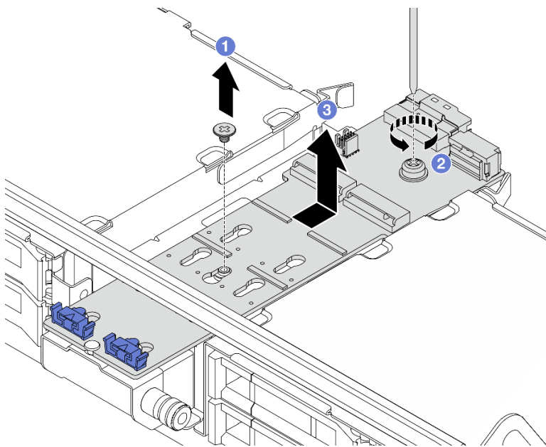
圖例 123. 從中間框架卸下 M.2 背板
