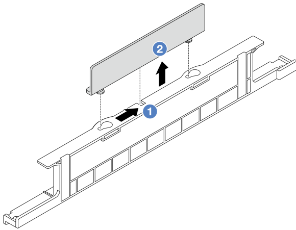
圖例 34. 卸下 2U 纜線壁托架
