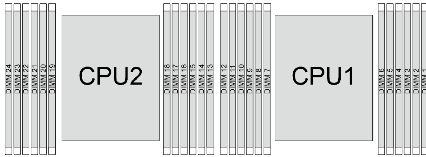
圖例 19. 記憶體模組和處理器佈置
