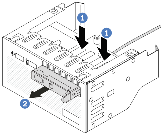
圖例 80. 卸下整合式診斷面板
