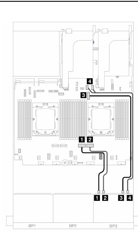
圖例 527. NVMe 纜線佈線
