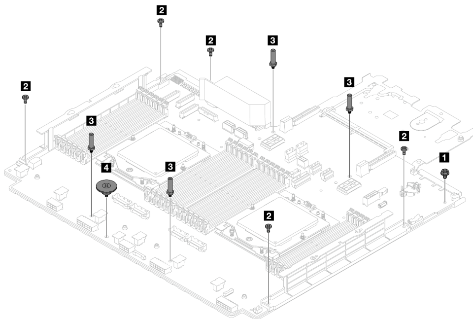
圖例 600. 從處理器板上卸下螺絲
