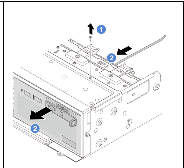
圖例 79. 具有整合式診斷面板的正面 I/O 模組
