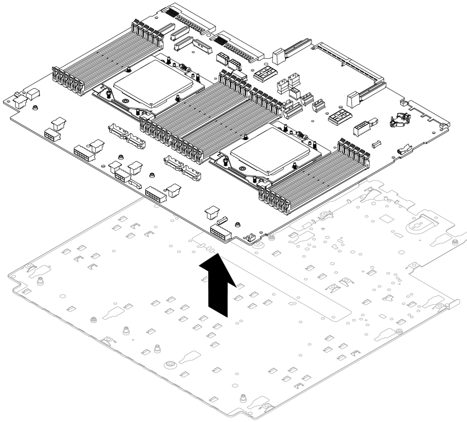
圖例 602. 將處理器板與支撐金屬板分開
