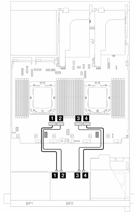
圖例 430. NVMe 纜線佈線
