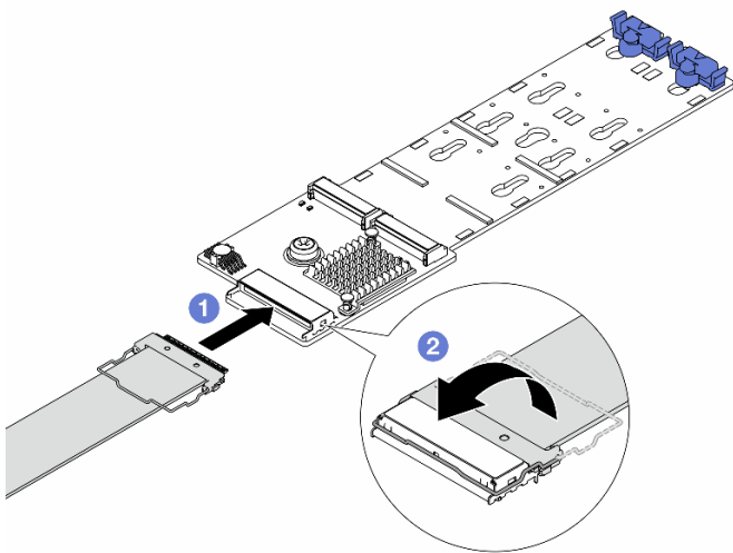
圖例 129. 將 M.2 纜線連接至 M.2 RAID SATA/NVME 2 機槽背板
