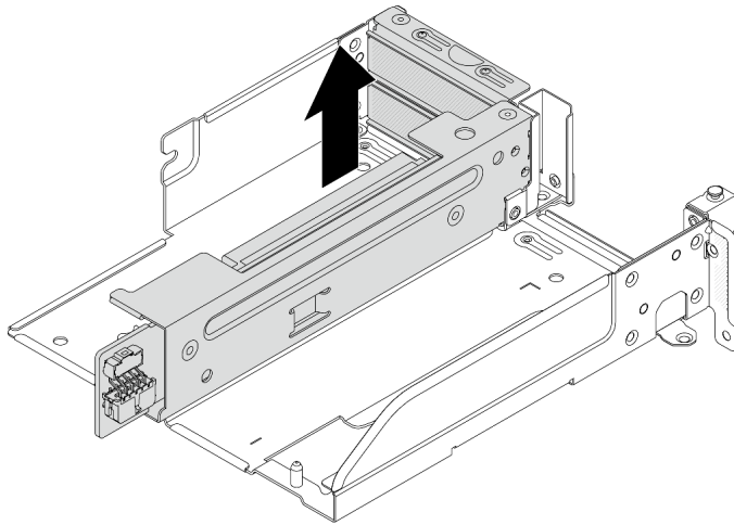
圖例 266. 卸下擴充卡 3/4 組件
