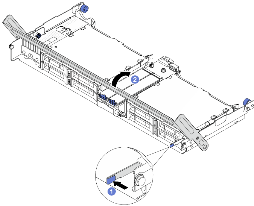
圖例 126. 關上中間框架的把手
