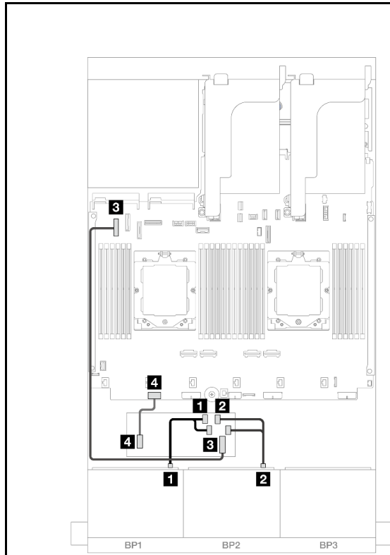
圖例 391. 安裝了兩個處理器的纜線佈線
