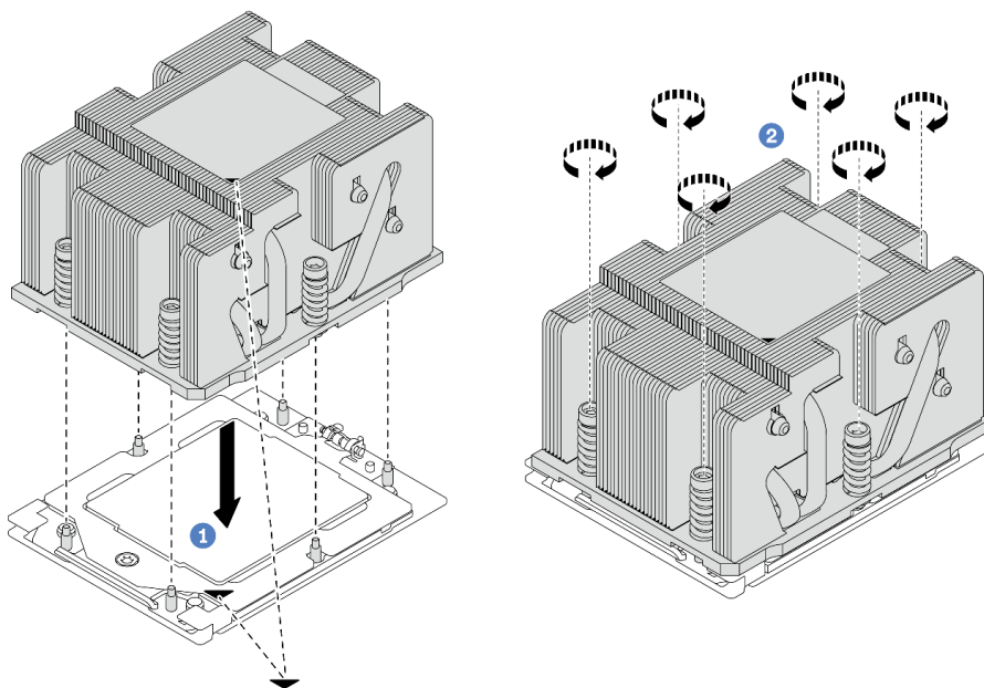
圖例 201. 安裝標準散熱槽
