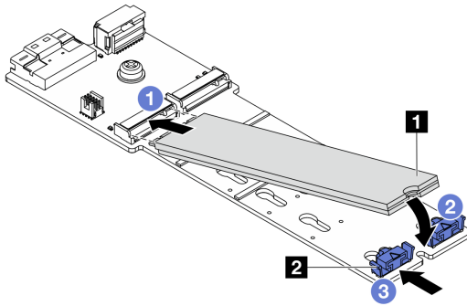
圖例 117. 安裝 M.2 硬碟
