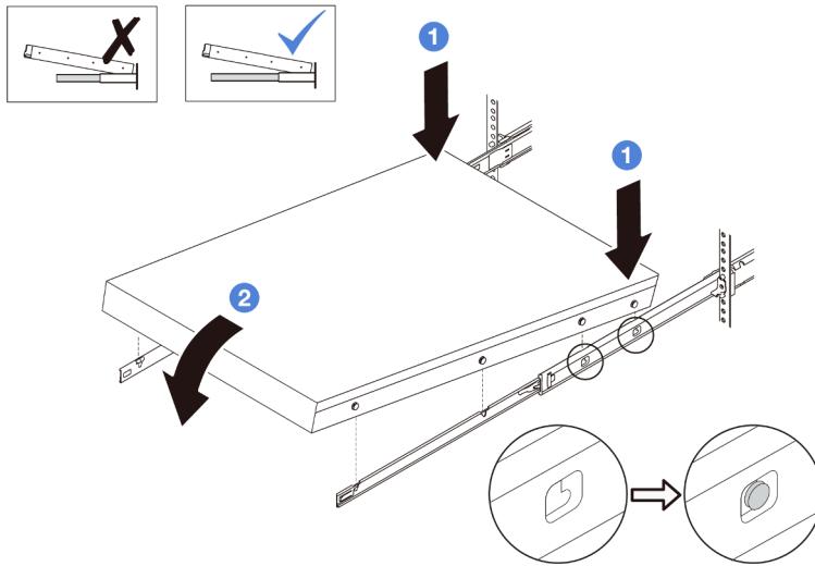
圖例 26. 將伺服器安裝到滑軌
