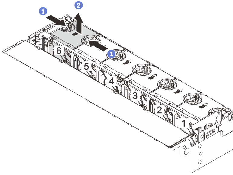
圖例 298. 卸下系統風扇
