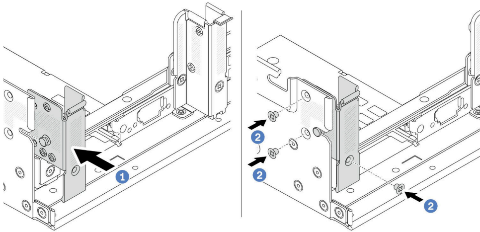
圖例 229. 安裝 A1 後壁托架 (左)
