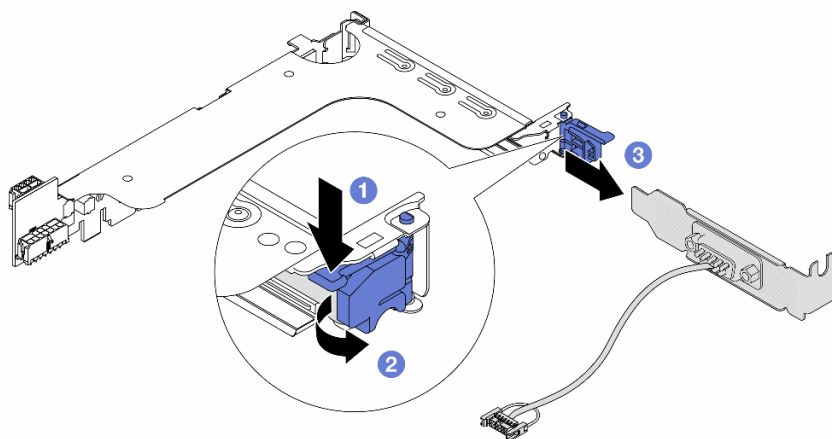
圖例 304. 卸下序列埠模組
