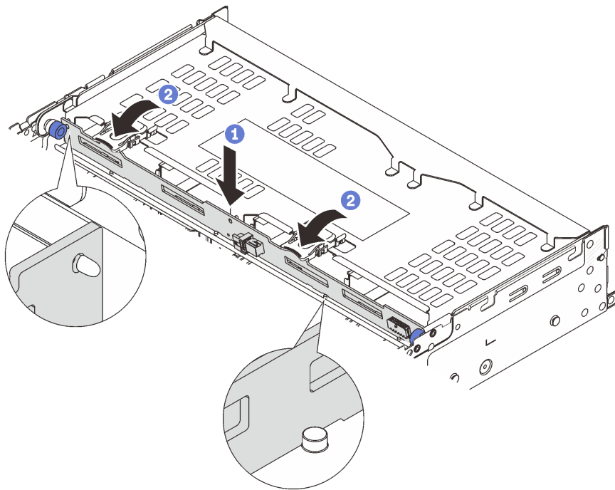
圖例 257. 安裝 4 x 3.5 吋後方硬碟背板
