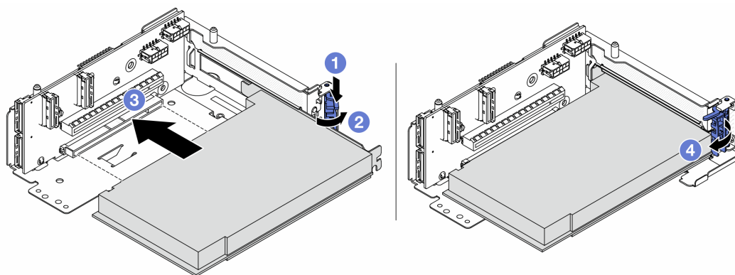
圖例 67. 將 PCIe 配接卡安裝到擴充卡 5 匣
