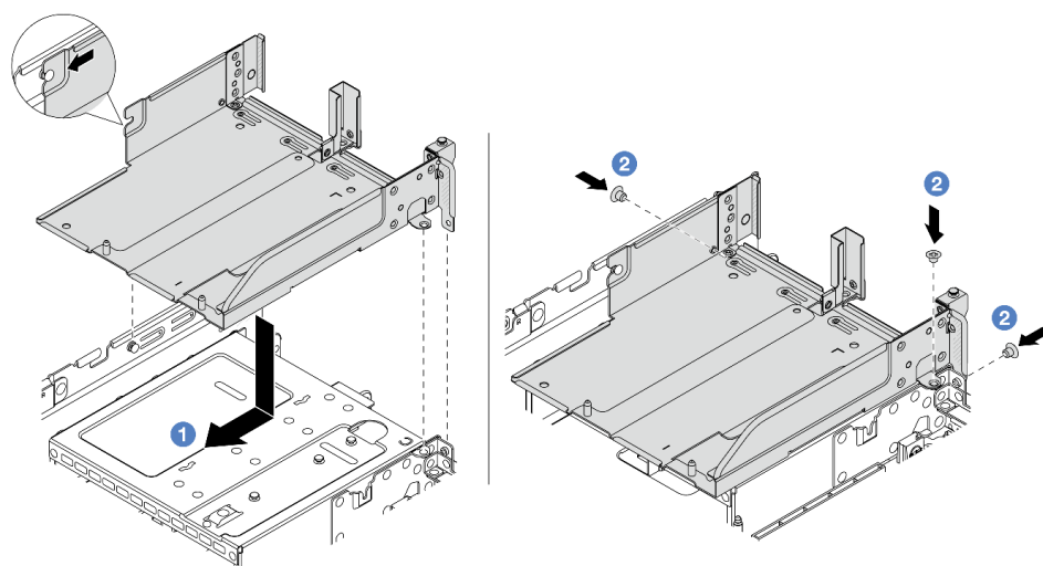
圖例 282. 安裝擴充卡匣托盤
