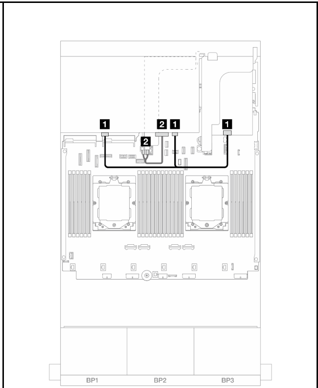
圖例 537. 後方背板纜線佈線
