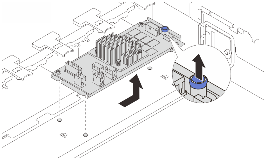
圖例 96. 卸下內部 CFF 配接卡
