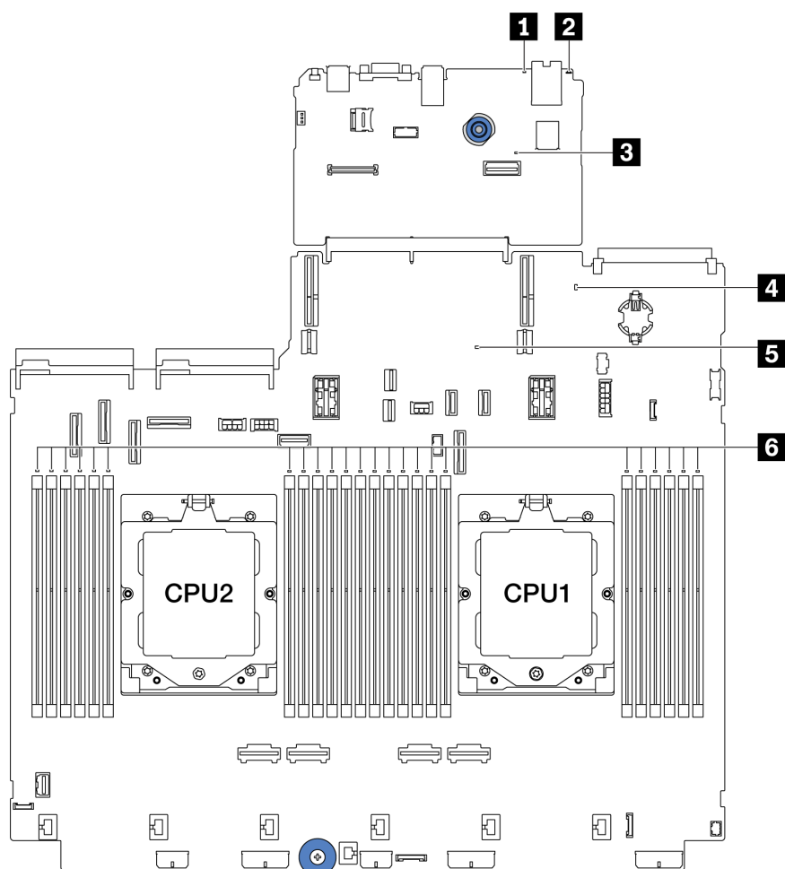
圖例 594. 主機板組件 LED
