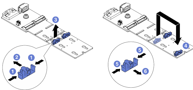
圖例 115. 調整 M.2 固定器
