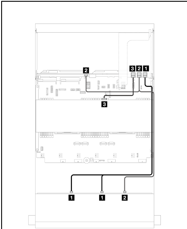
圖例 565. 前方/後方背板信號線佈線
