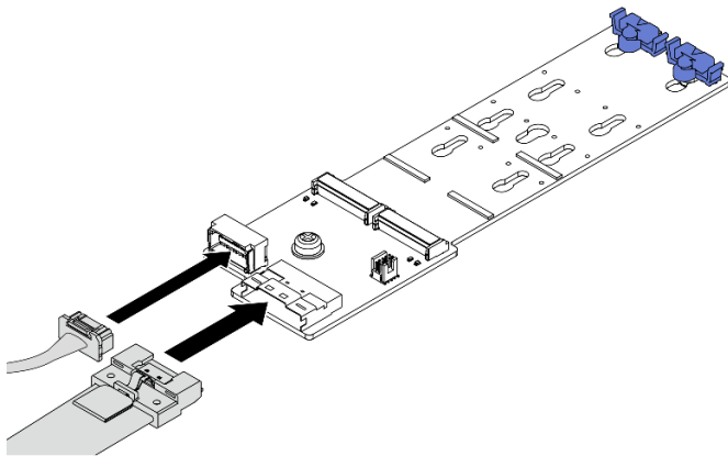
圖例 127. 將 M.2 纜線連接至 M.2 x4 非 RAID SATA/NVMe 2 機槽背板
