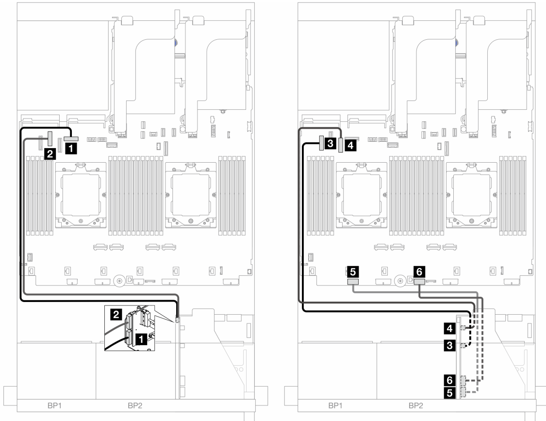
圖例 355. 不含擴充卡 3/4 的配置的纜線佈線
