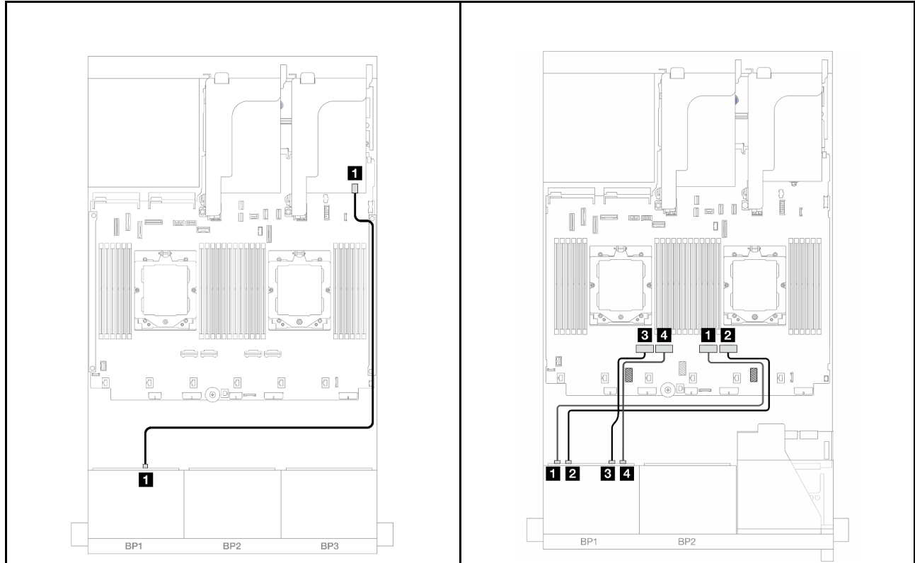
圖例 370. SAS/SATA 纜線佈線
