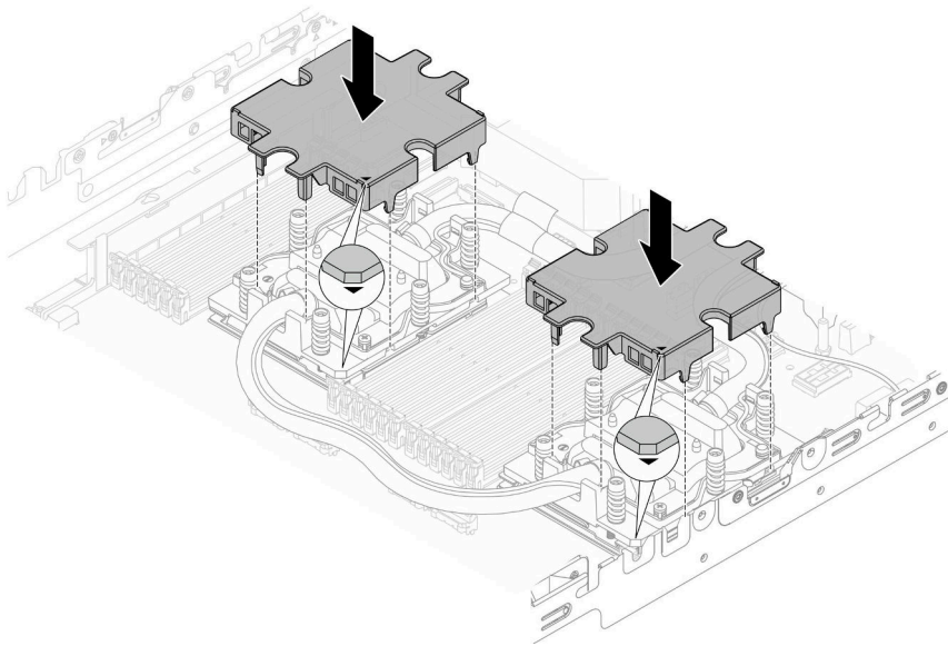
圖例 109. 安裝水冷板蓋
