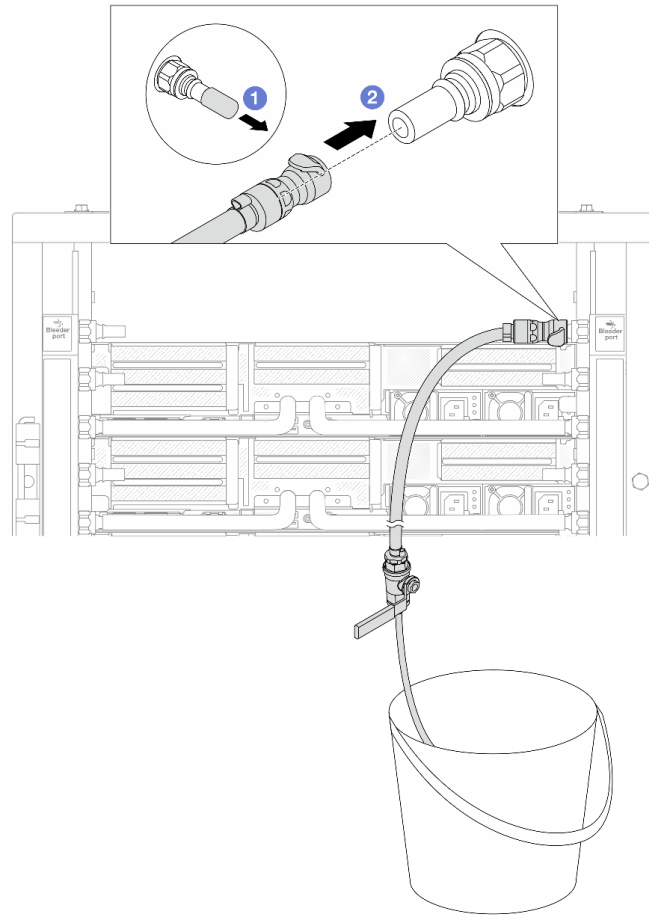
圖例 174. 在回流側安裝洩放套件
