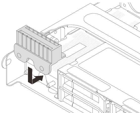
圖例 225. 安裝橡膠
