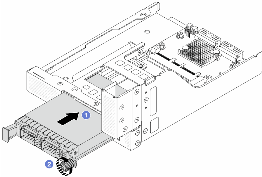
圖例 45. 安裝 OCP 模組
