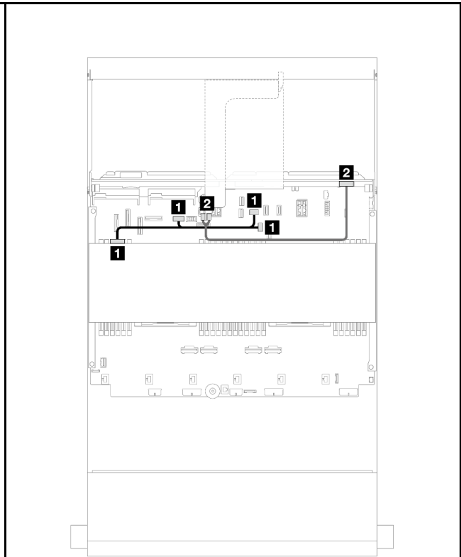
圖例 564. 中間/後方背板電源線佈線
