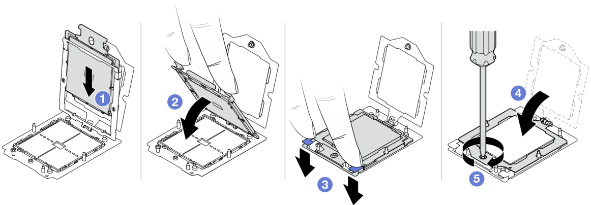
圖例 199. 安裝處理器
