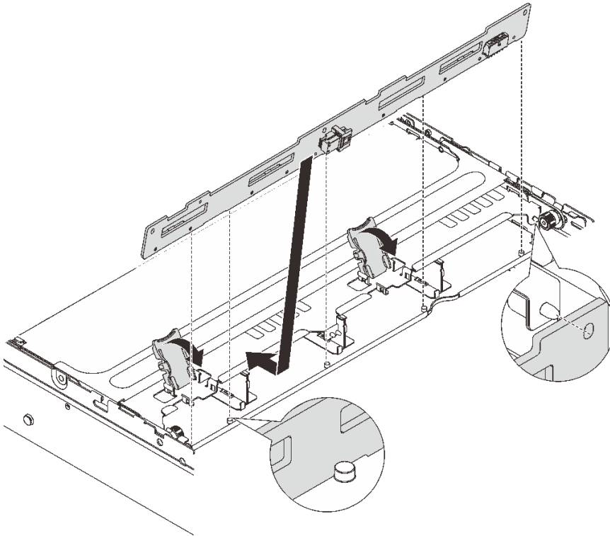
圖例 187. 安裝中間 3.5 吋硬碟背板
