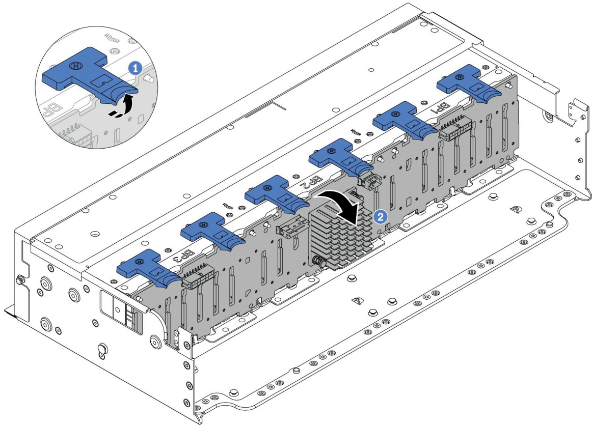
圖例 71. 卸下 24 機槽硬碟背板
