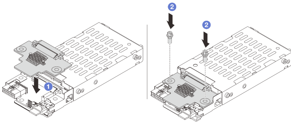
圖例 238. 安裝 7 公釐硬碟背板 (頂端)
