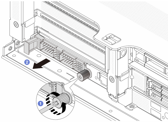
圖例 260. 卸下背面 OCP 模組
