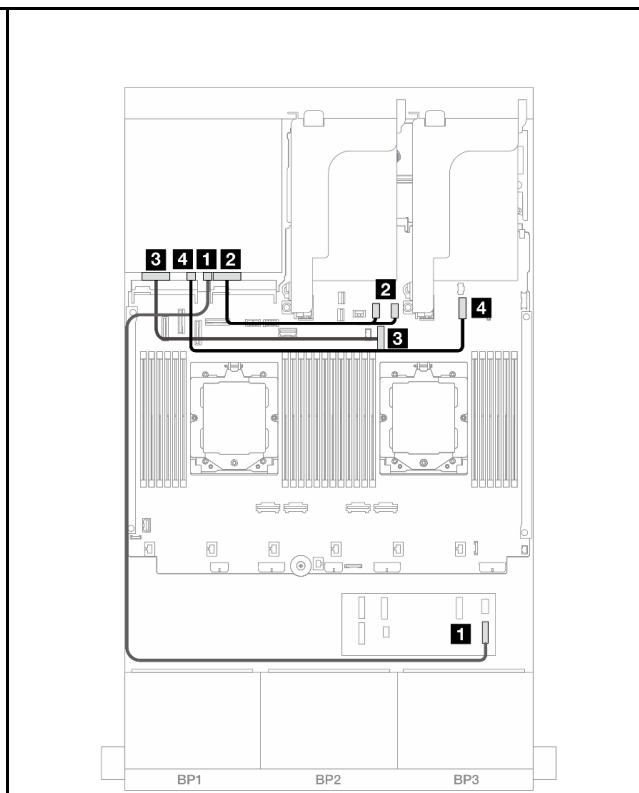
圖例 456. 安裝了一個處理器的纜線佈線
