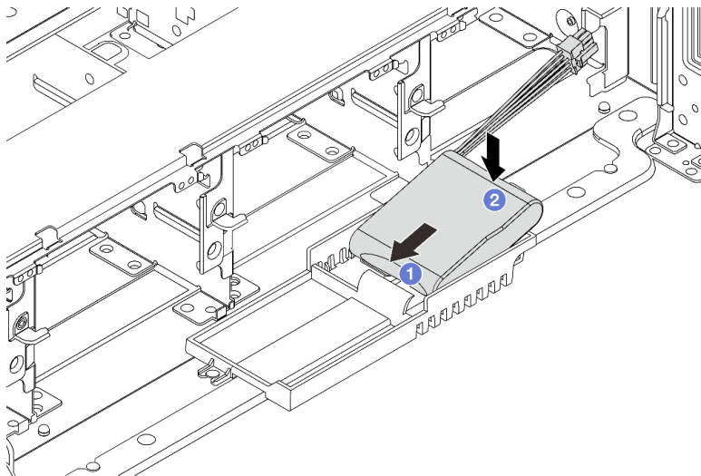
圖例 217. 將 RAID 快閃記憶體電源模組安裝在超級電容固定器上
