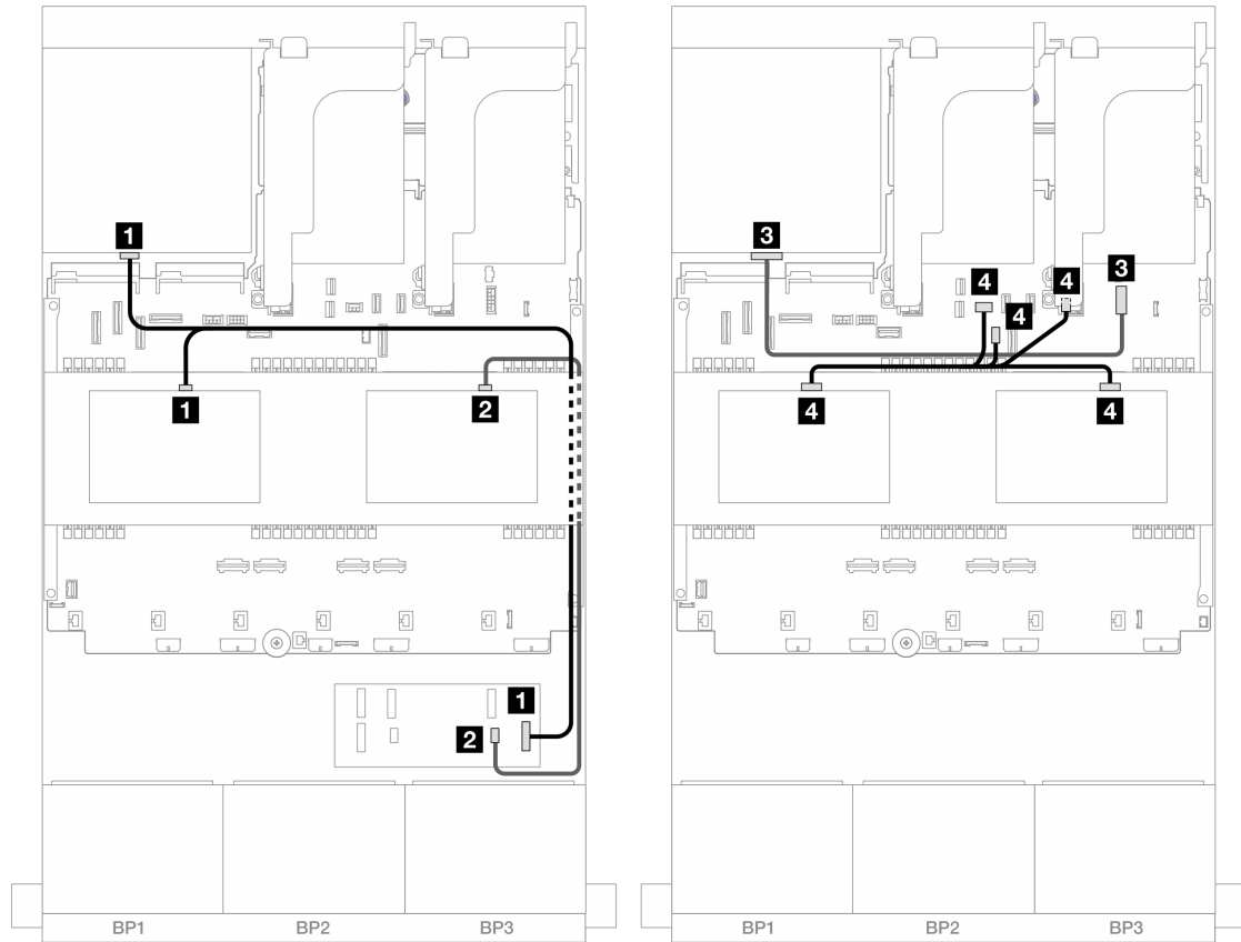
圖例 483. 中間/後方背板纜線佈線
