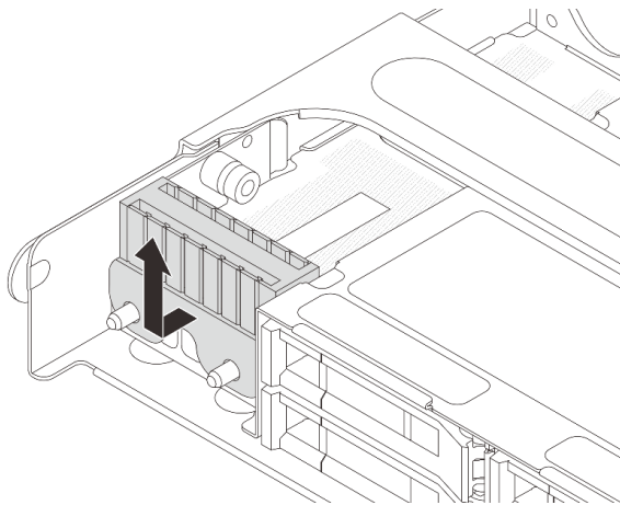
圖例 220. 卸下橡膠
