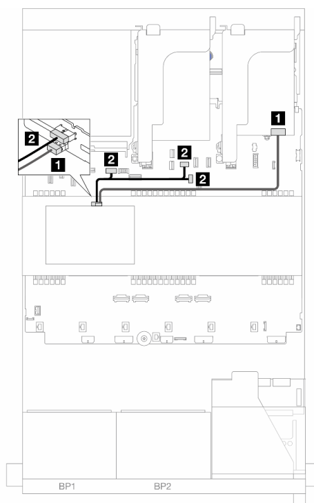
圖例 396. 中間背板纜線佈線
