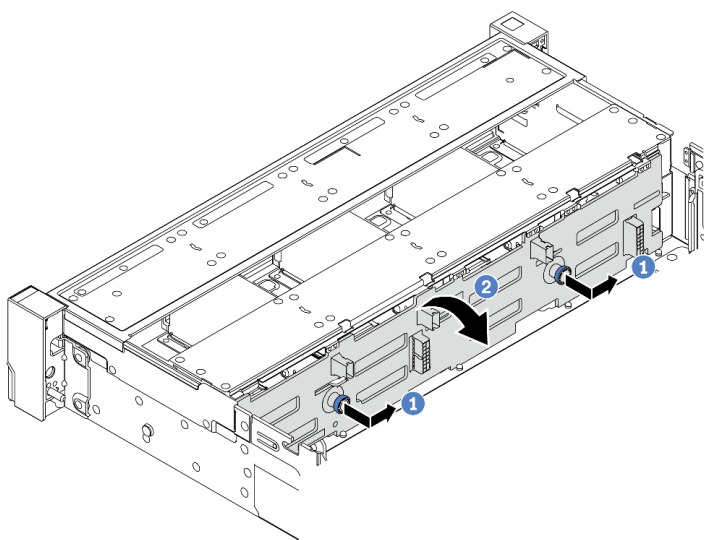
圖例 75. 卸下 3.5 吋硬碟背板
