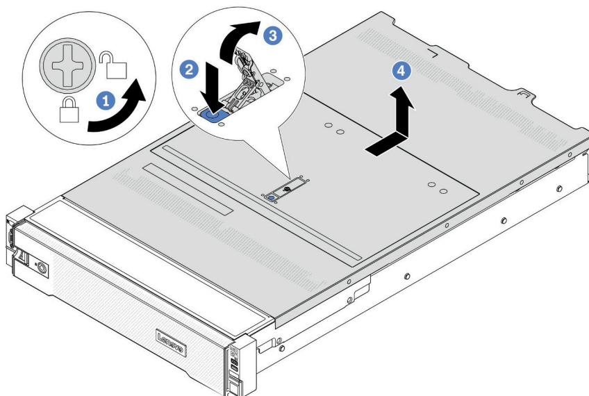
圖例 309. 卸下上蓋
