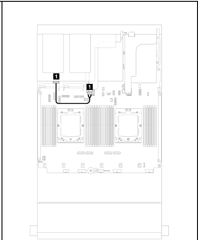
圖例 552. 後方背板電源線佈線
