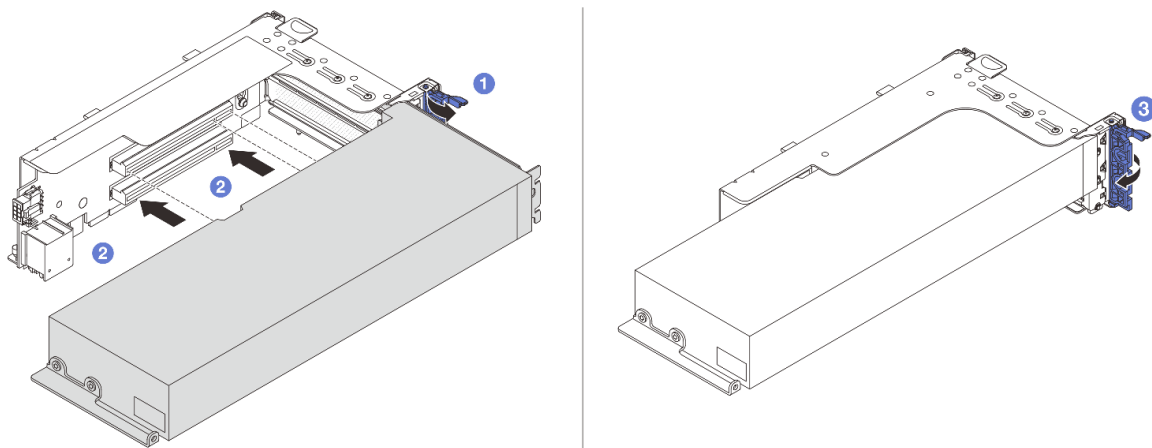
圖例 91. 安裝 GPU 配接卡
