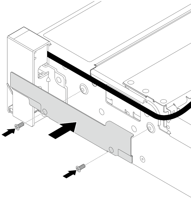
圖例 209. 安裝纜線固定夾
