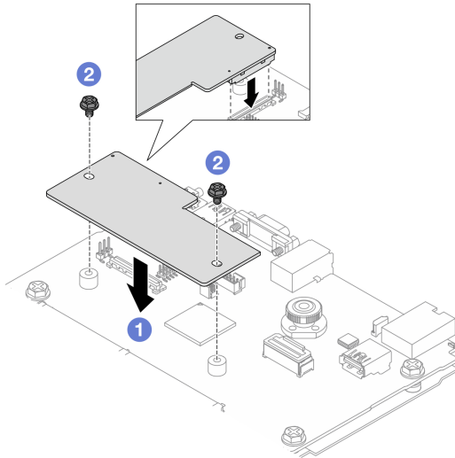
圖例 291. 安裝韌體和 RoT 安全模組
