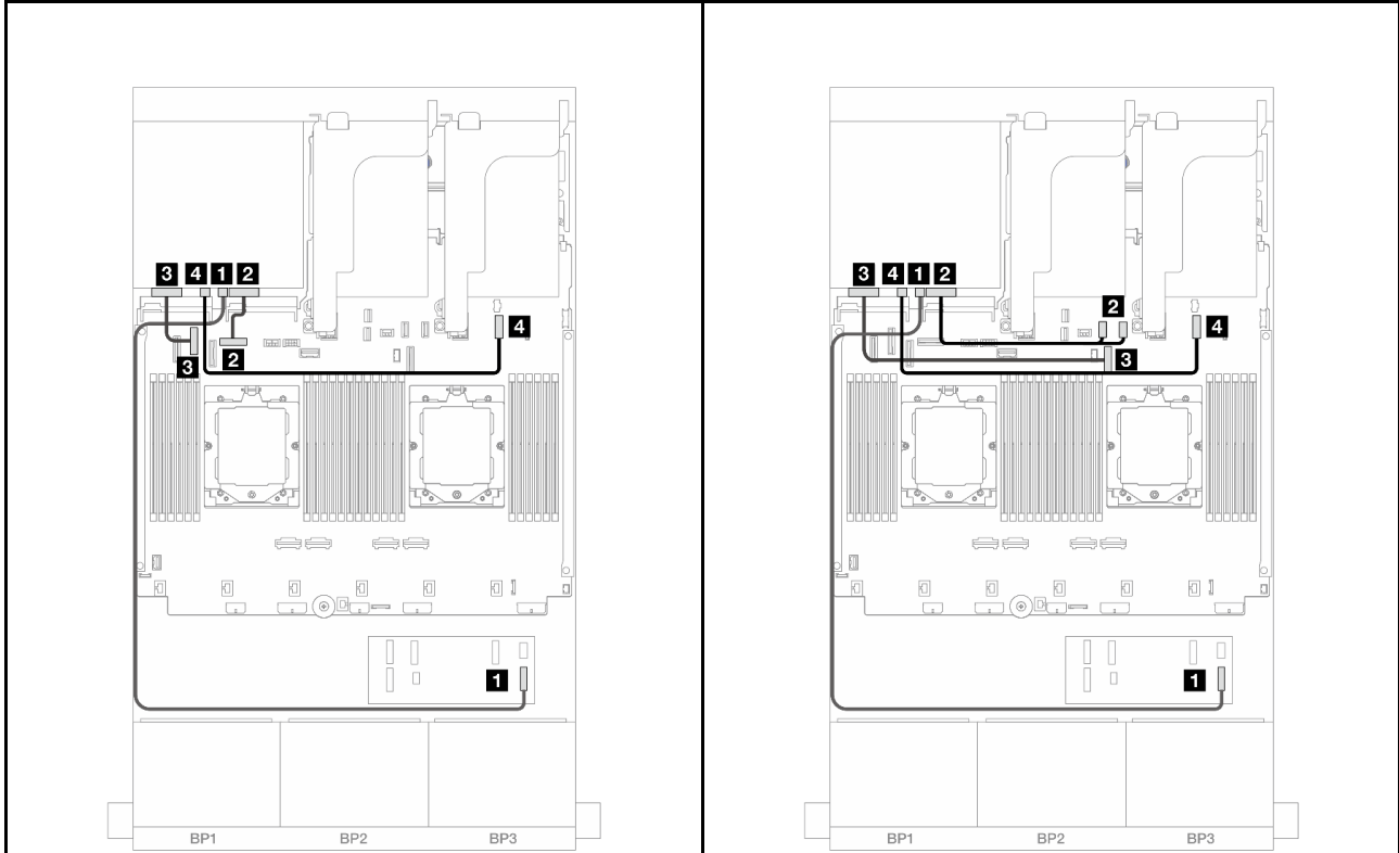
圖例 451. 安裝了兩個處理器的纜線佈線
