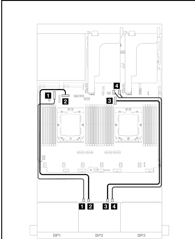
圖例 407. 安裝了兩個處理器的纜線佈線
