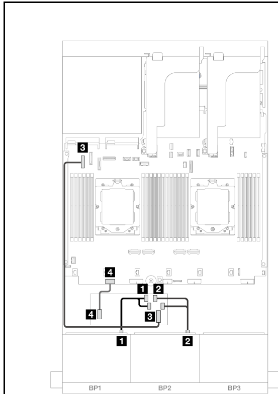
圖例 520. 纜線佈線至 CFF 配接卡
