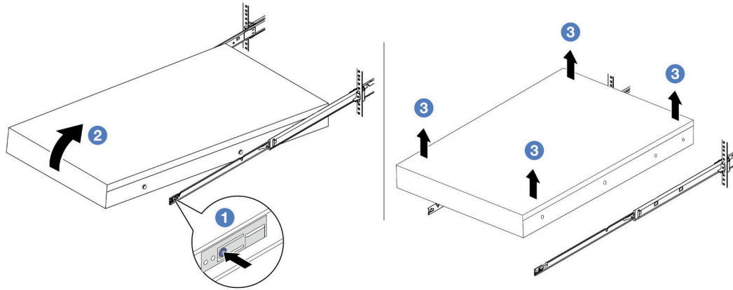
圖例 23. 從機架卸下伺服器。
