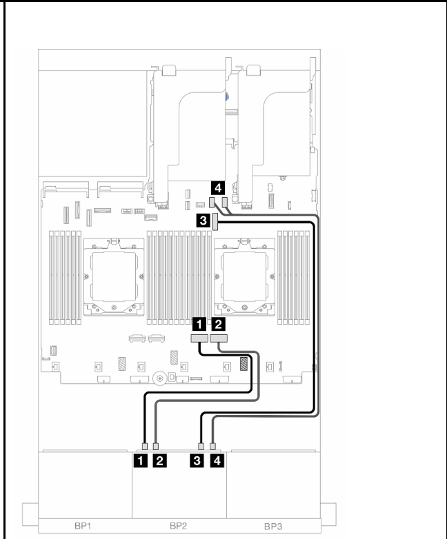
圖例 408. 安裝了一個處理器的纜線佈線
