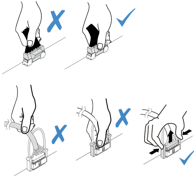
圖例 95. 從主機板組件拔掉纜線
