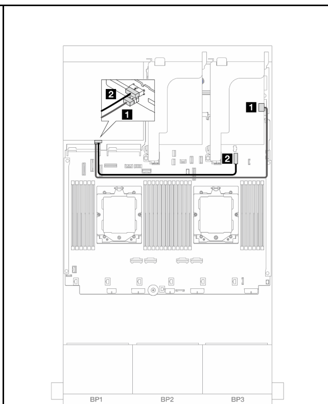
圖例 441. 後方背板纜線佈線
