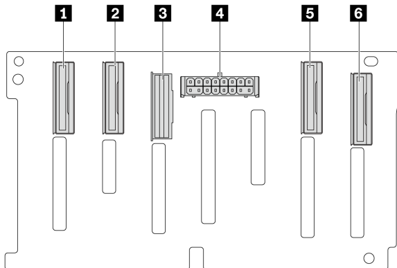
圖例 312. 8 x 2.5 吋 AnyBay 背板接頭
