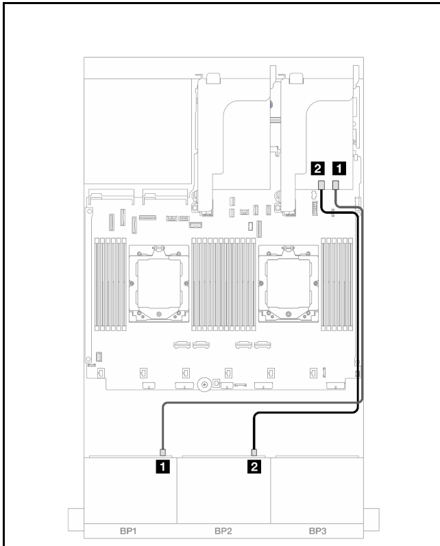
圖例 397. 前方背板纜線佈線
