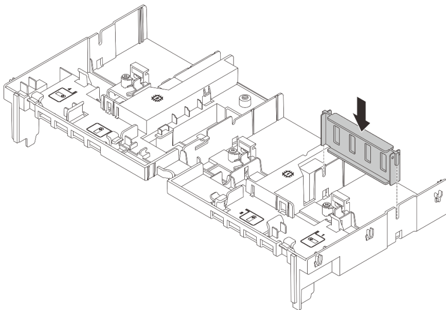
圖例 94. 安裝 GPU 空氣擋板填充板
