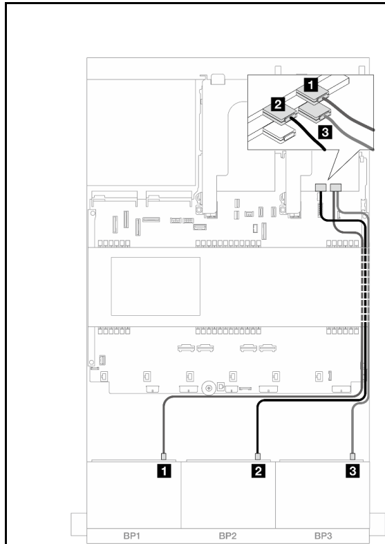
圖例 475. 前方背板纜線佈線
