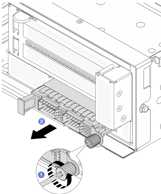
圖例 50. 卸下正面 OCP 模組
