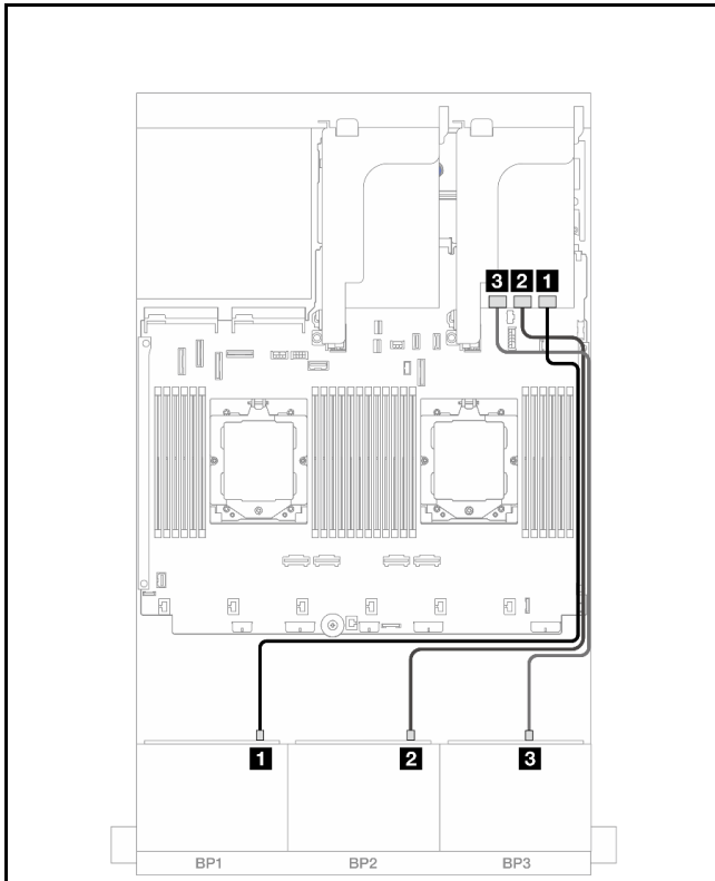
圖例 508. SAS/SATA 纜線佈線
