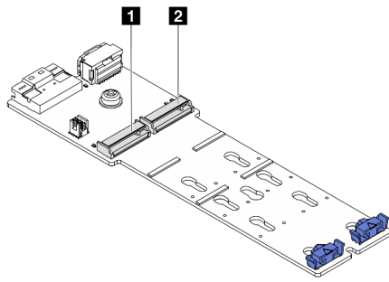
圖例 116. M.2 硬碟插槽
