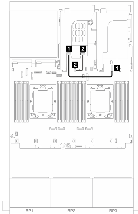
圖例 328. 7 公釐 RAID SATA/NVMe 2 機槽背板的纜線佈線
