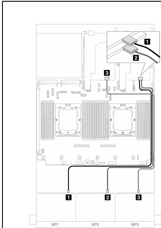
圖例 506. SAS/SATA 纜線佈線
