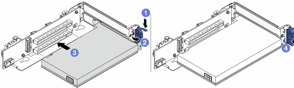
圖例 278. 將 PCIe 配接卡安裝到擴充卡 3 組件
