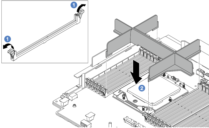
圖例 197. 安裝處理器填充板
