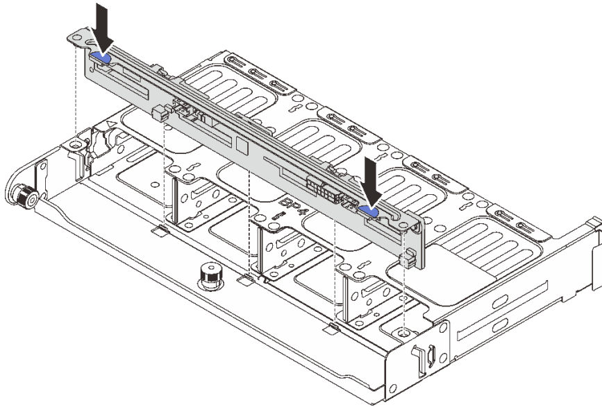
圖例 249. 安裝 8 x 2.5 吋後方硬碟背板
