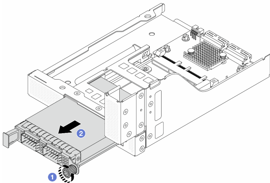
圖例 54. 卸下 OCP 模組
