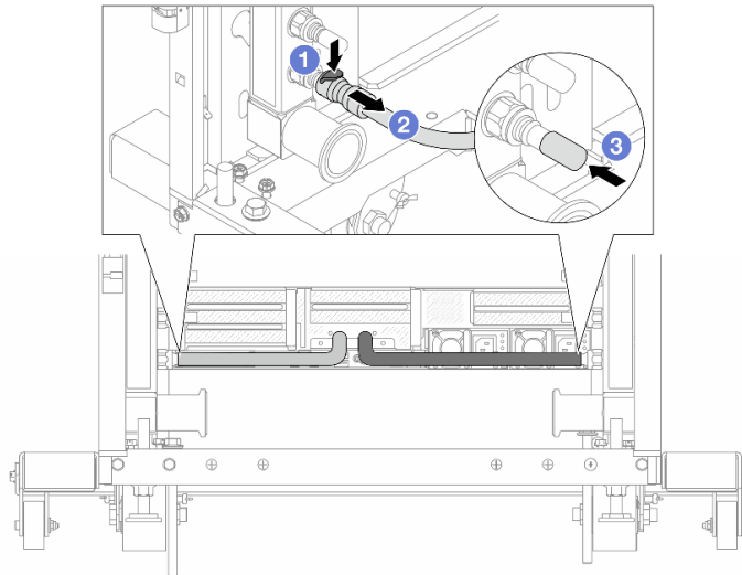
圖例 139. 移除 quick connect 插頭
