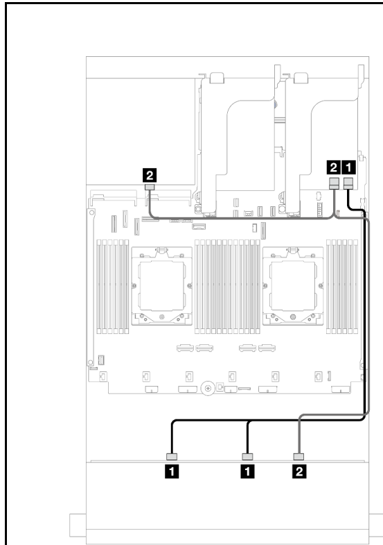
圖例 553. 前方/後方背板信號線佈線
