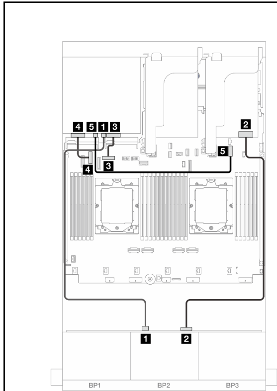
圖例 534. 安裝了兩個處理器的纜線佈線
