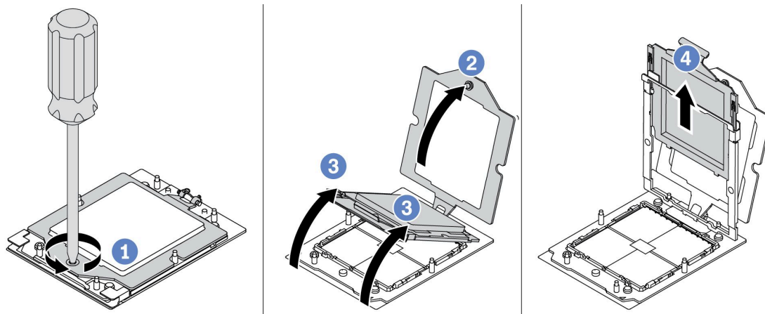
圖例 196. 卸下處理器
