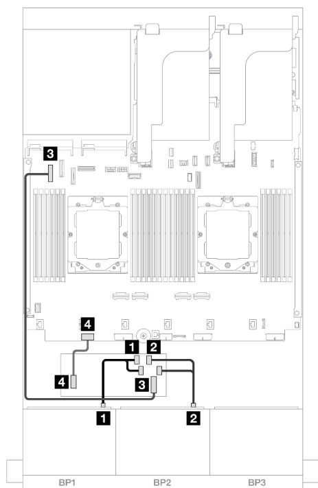
圖例 530. 纜線佈線至 CFF 配接卡
