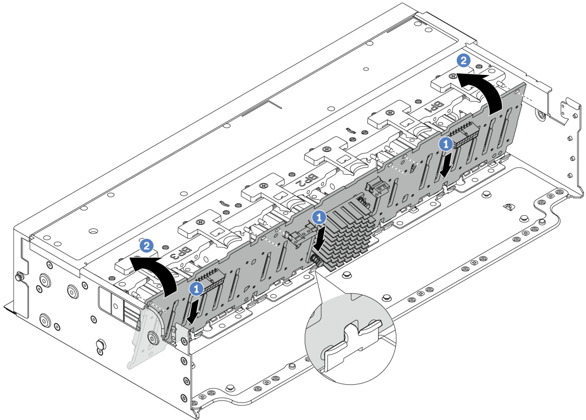
圖例 74. 安裝 24 機槽擴充器背板
