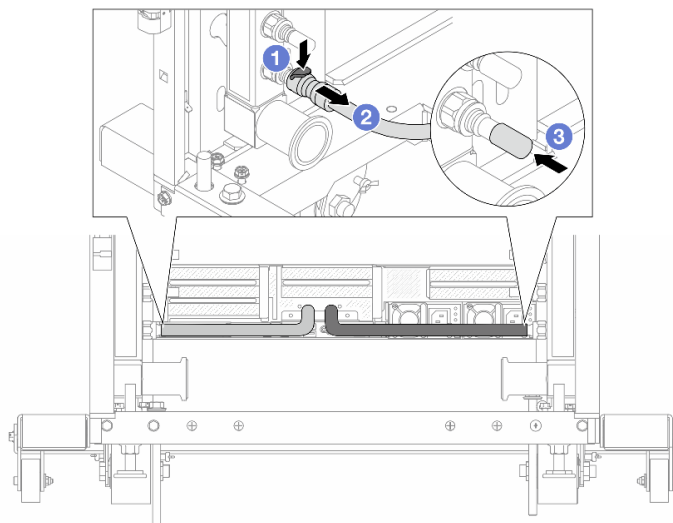
圖例 161. 移除 quick connect 插頭
