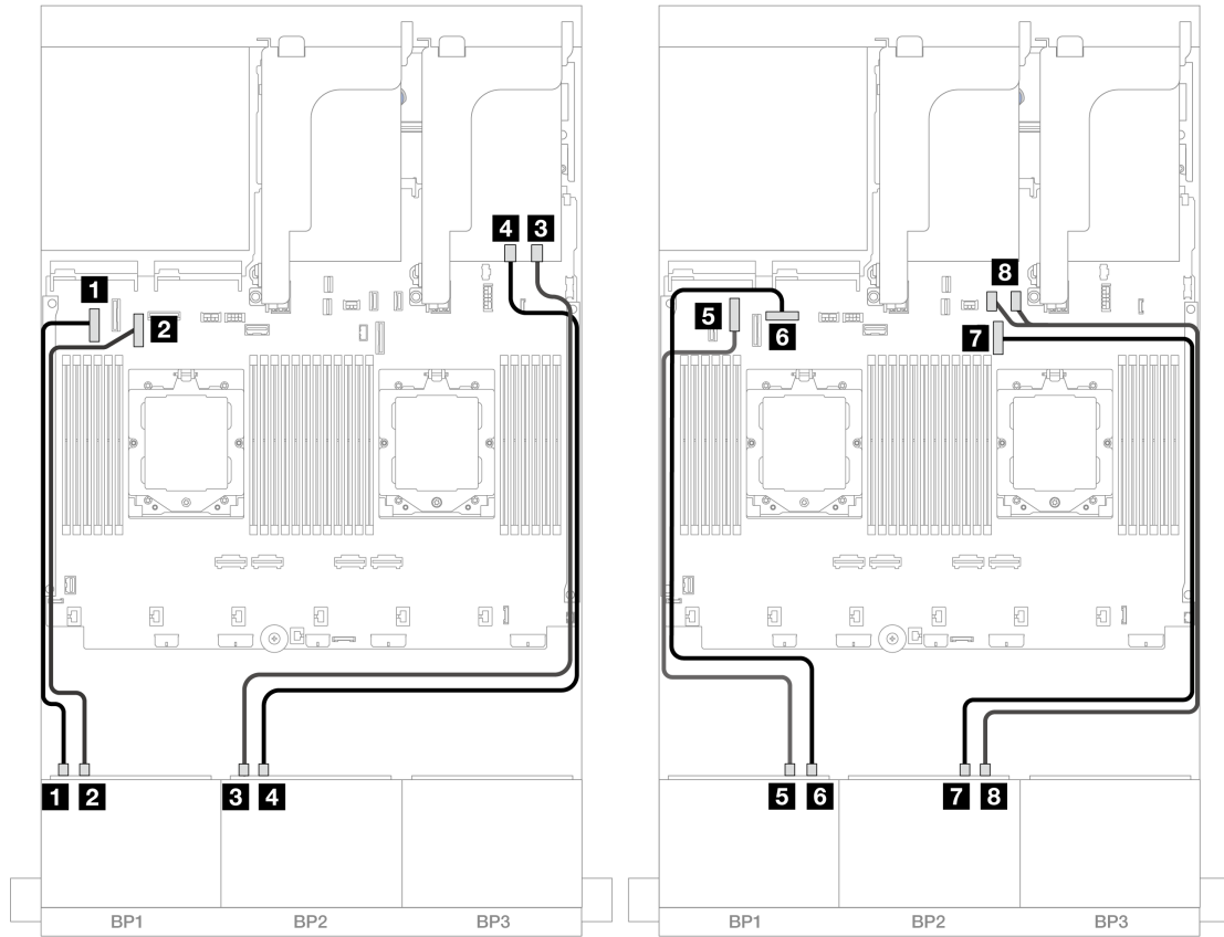
圖例 405. NVMe 纜線佈線至機載接頭和重定時器卡
