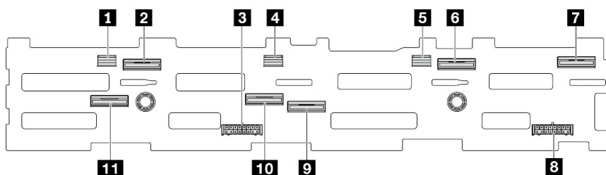
圖例 317. 12 x 3.5 吋 AnyBay 背板接頭
