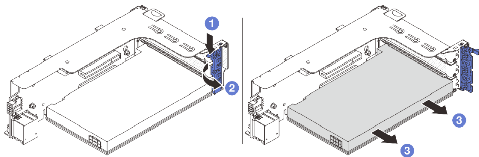
圖例 268. 從擴充卡 1 或 2 組件卸下 PCIe 配接卡
