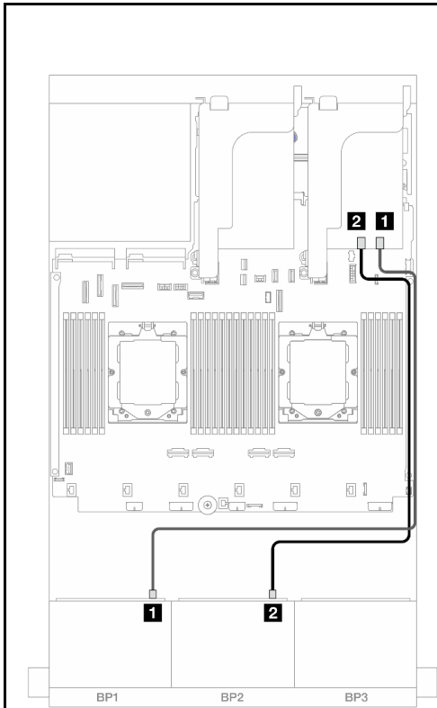
圖例 526. SAS/SATA 纜線佈線
