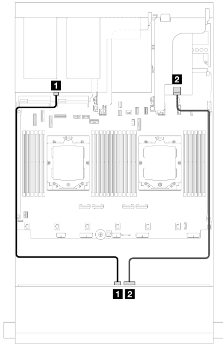
圖例 580. 前方/後方背板信號線佈線
