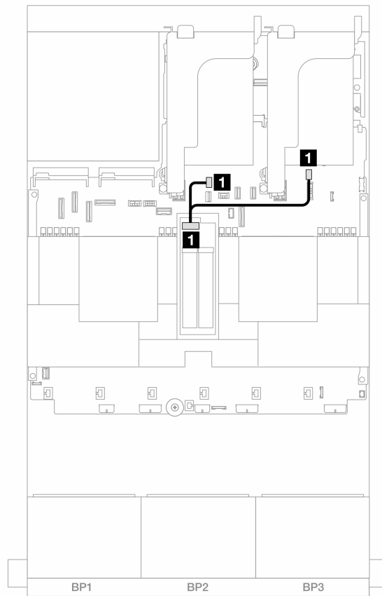
圖例 338. M.2 RAID SATA/NVME 2 機槽背板的纜線佈線
