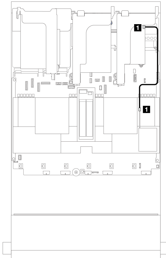
圖例 345. RAID 快閃記憶體電源模組的纜線佈線
