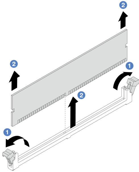
圖例 179. 卸下記憶體模組
