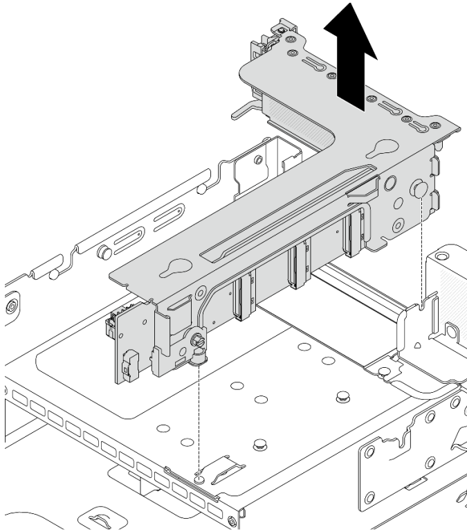
圖例 265. 卸下擴充卡 3 組件
