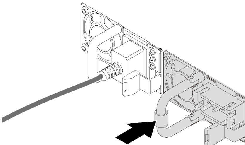
圖例 192. 安裝電源供應器
