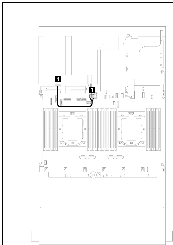
圖例 549. 安裝了兩個處理器的纜線佈線
