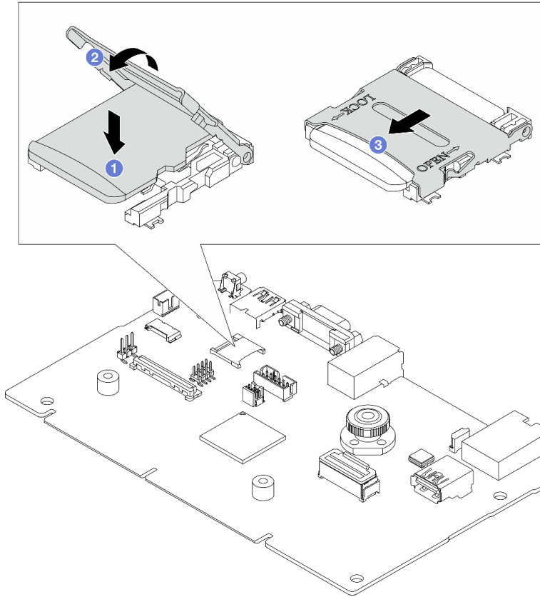
圖例 295. 安裝 MicroSD 卡
