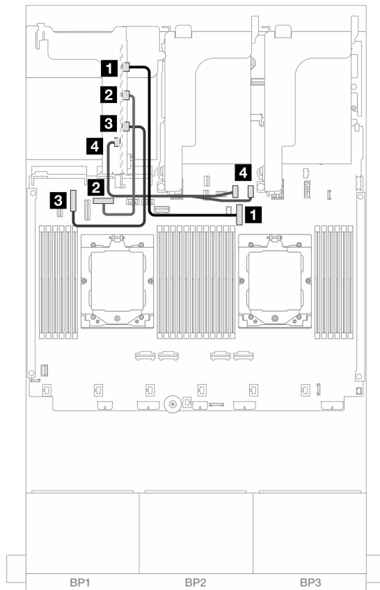
圖例 349. x16/x16 Gen 4 PCIe 擴充卡 3 的信號線連接
