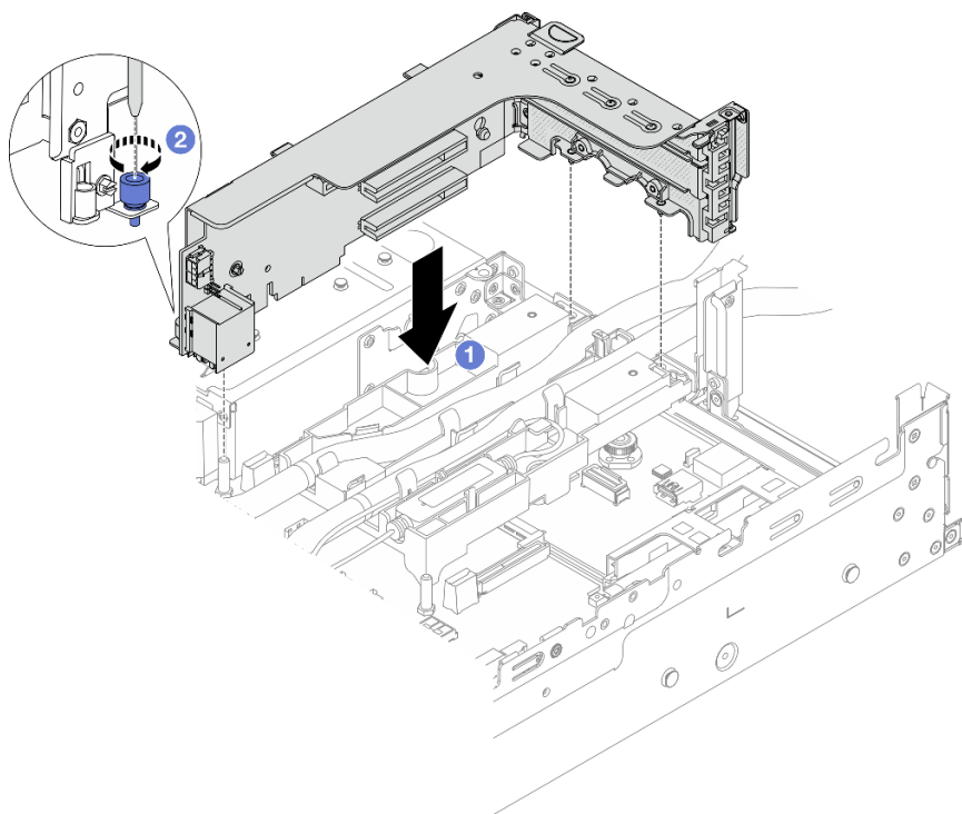
圖例 113. 安裝 3FH 擴充卡匣
