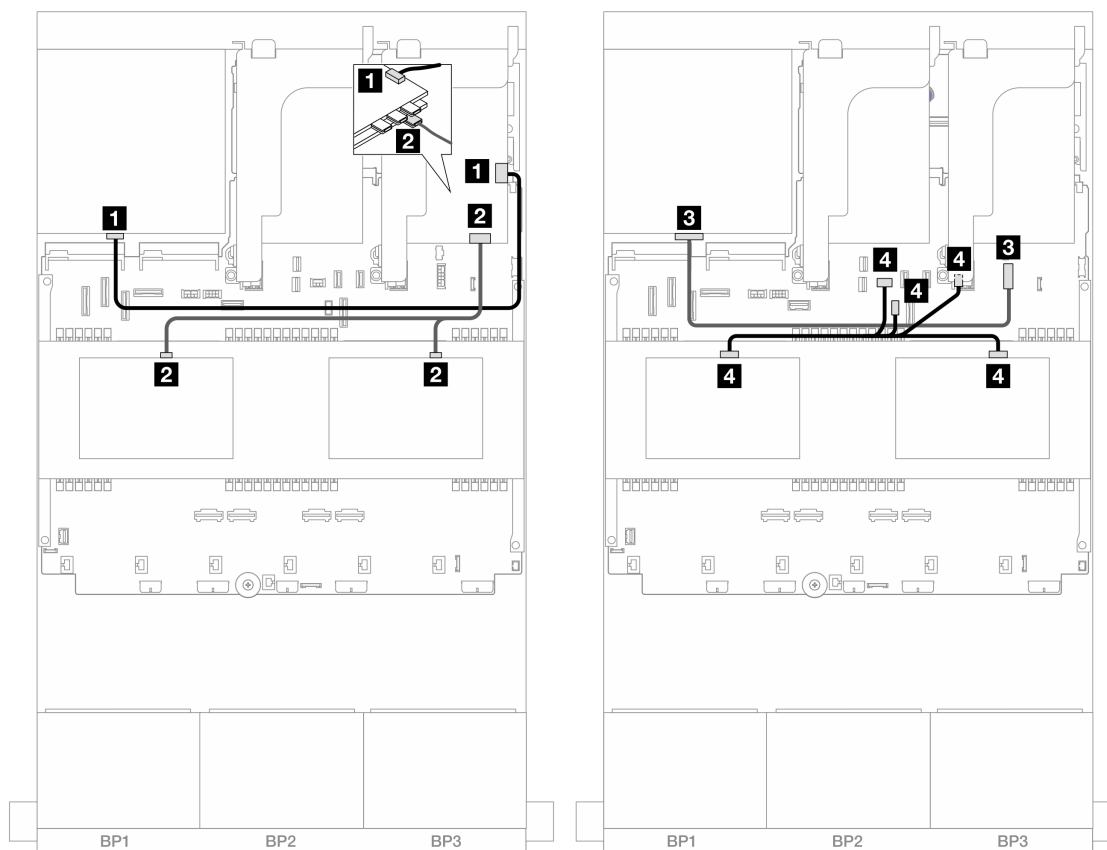
圖例 478. 中間/後方背板纜線佈線
