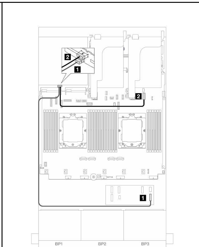
圖例 443. 後方背板纜線佈線
