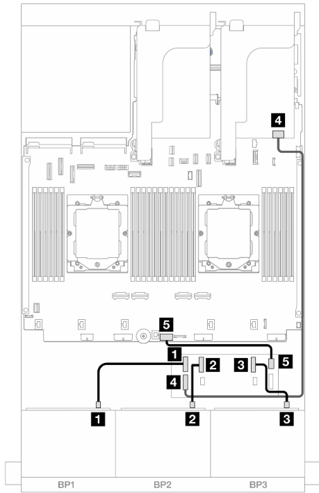
圖例 464. 前方背板纜線佈線
