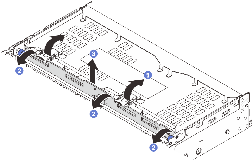
圖例 256. 卸下 4 x 3.5 吋後方硬碟背板
