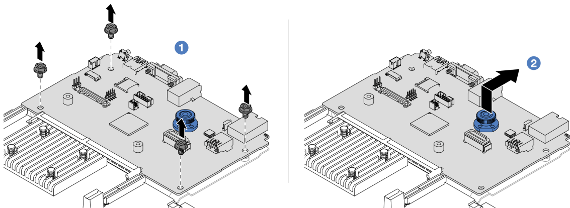
圖例 599. 將系統 I/O 板與處理器板分開
