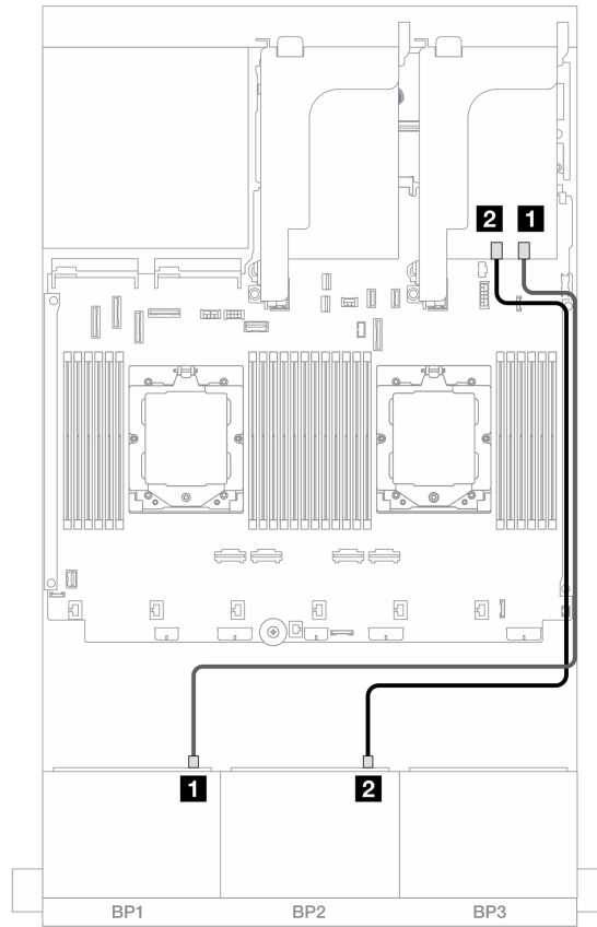
圖例 390. SAS/SATA 纜線佈線至 16i RAID/HBA 配接卡
