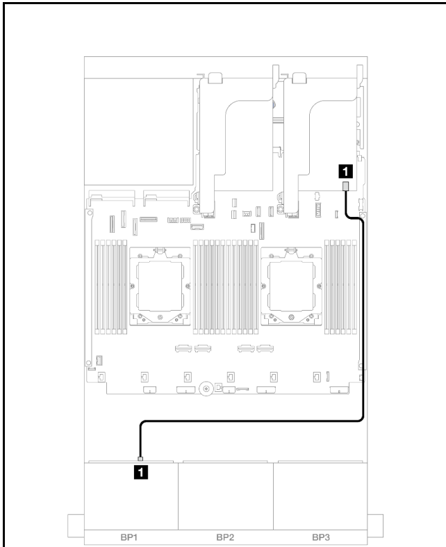
圖例 382. SAS/SATA 纜線佈線
