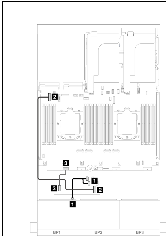
圖例 363. 安裝了兩個處理器的纜線佈線
