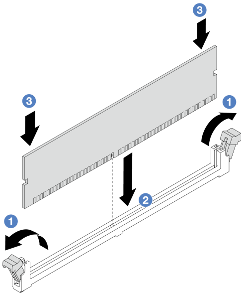
圖例 180. 安裝記憶體模組
