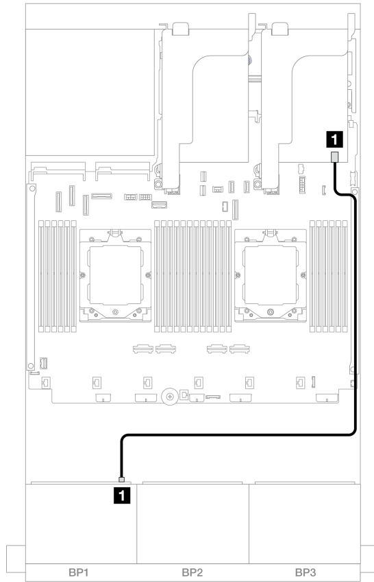
圖例 362. SAS/SATA 纜線佈線至 8i/16i RAID/HBA 配接卡
