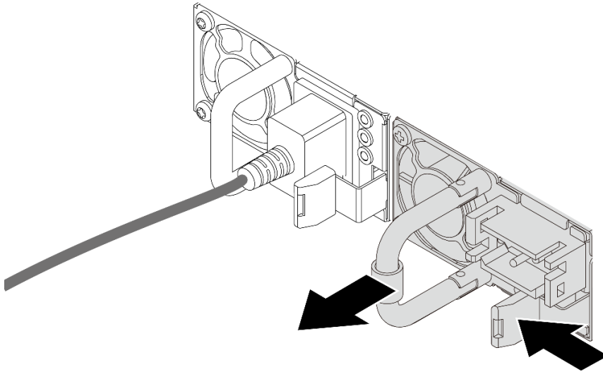
圖例 190. 卸下電源供應器
