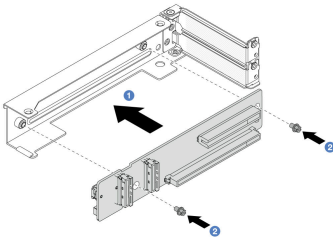
圖例 276. 將擴充卡安裝到 4LP 擴充卡 3/4 匣
