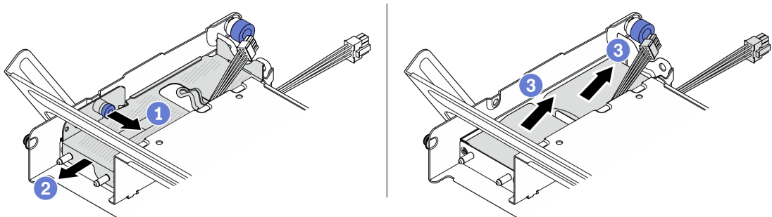
圖例 222. 從中間框架卸下 RAID 快閃記憶體電源模組
