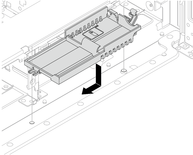
圖例 216. 安裝超級電容固定器
