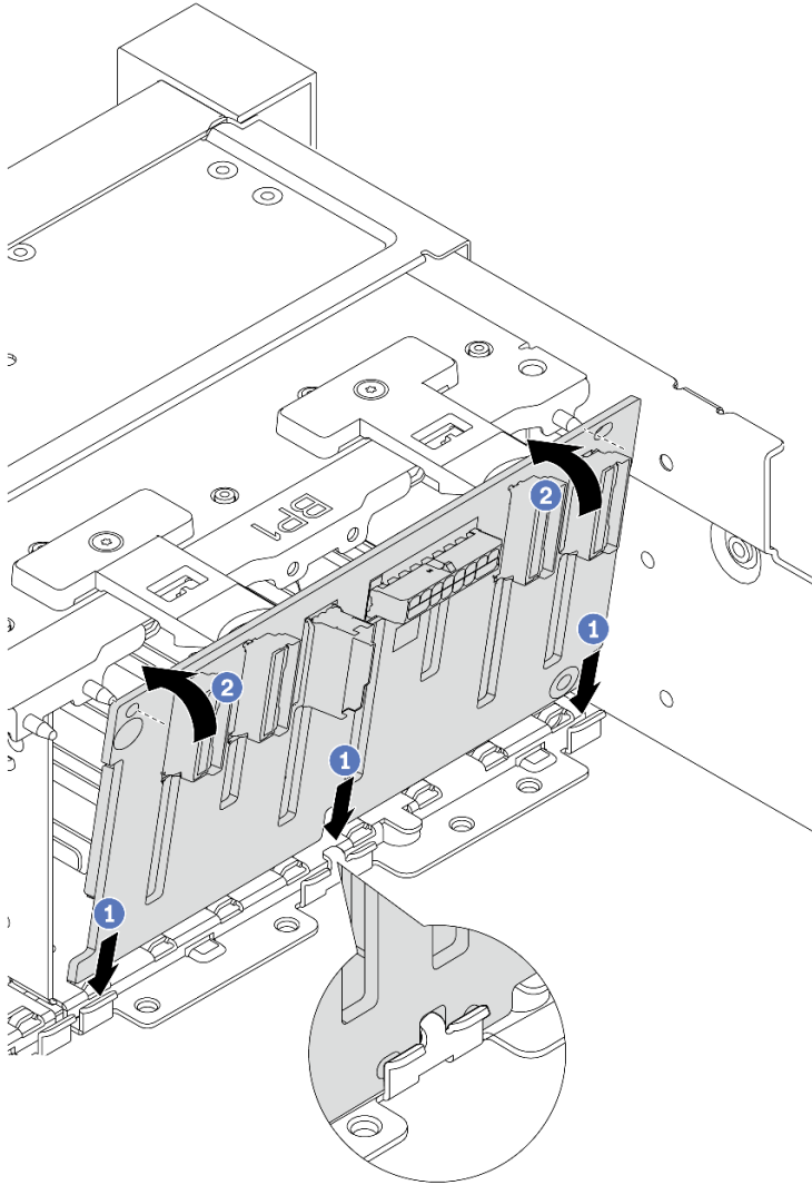
圖例 73. 安裝 8 機槽硬碟背板
