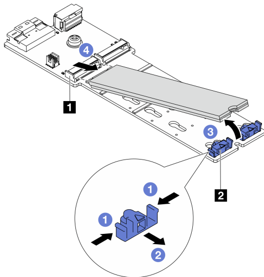
圖例 114. 卸下 M.2 硬碟
