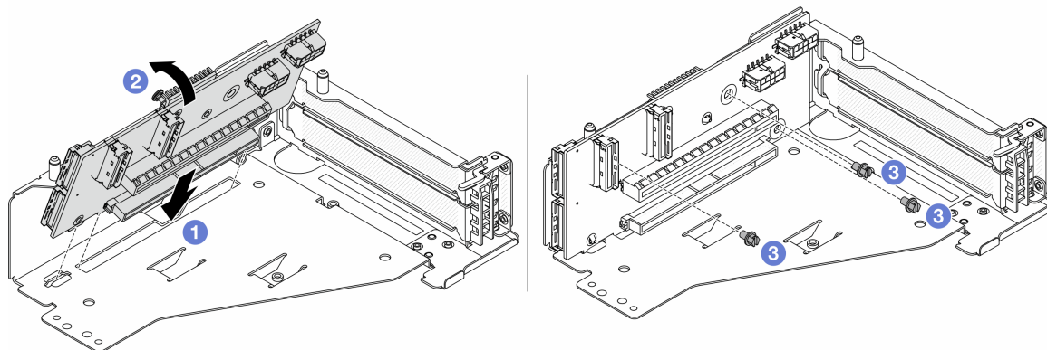
圖例 66. 安裝擴充卡
