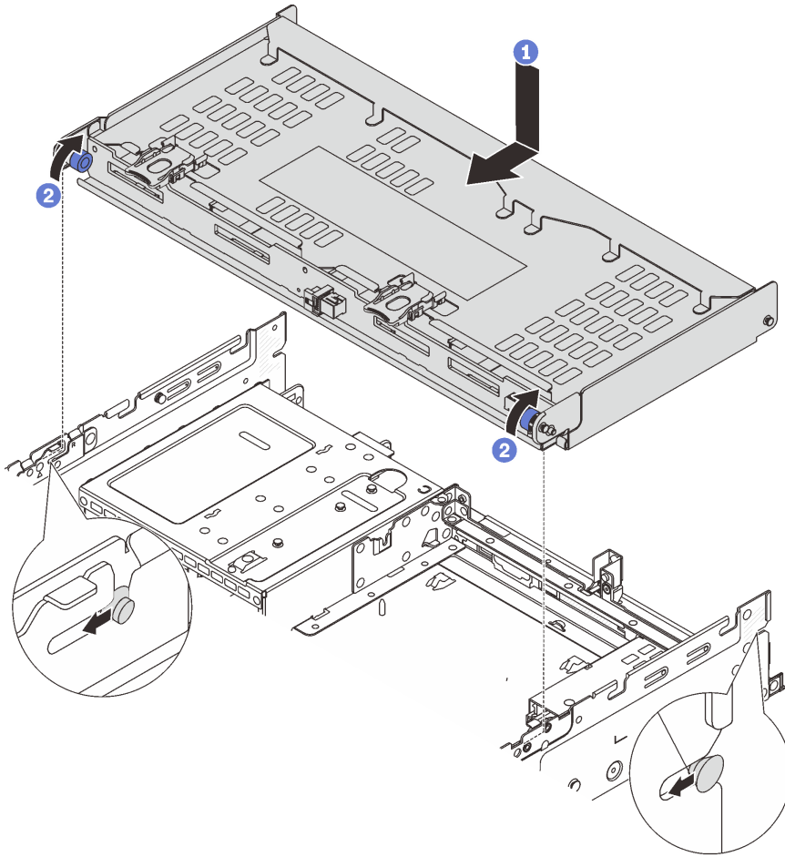
圖例 258. 安裝 4 x 3.5 吋背面框架
