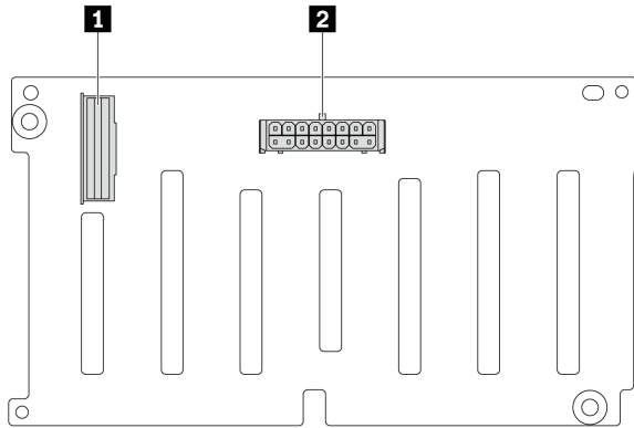
圖例 311. 8 x 2.5 吋 SAS/SATA 背板接頭
