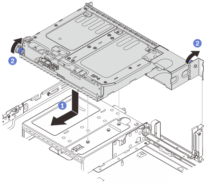
圖例 254. 安裝 2 x 3.5 吋背面框架
