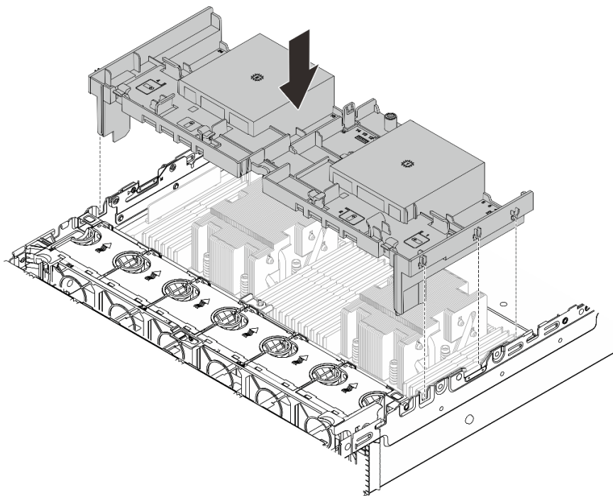
圖例 33. 安裝空氣擋板
