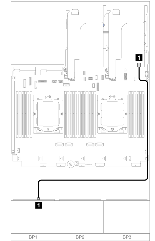
圖例 377. SAS/SATA 纜線佈線至 8i RAID/HBA 配接卡
