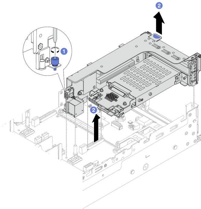
圖例 232. 卸下 2FH + 7 公釐 SSD 擴充卡匣
