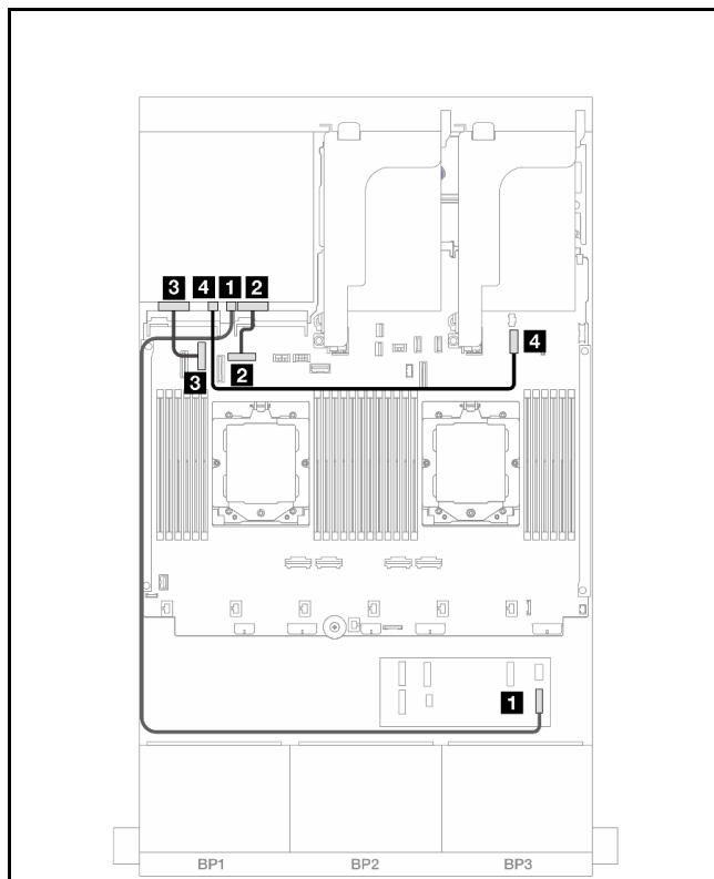
圖例 455. 安裝了兩個處理器的纜線佈線
