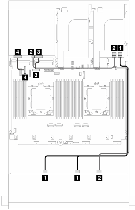
圖例 555. 安裝了兩個處理器的纜線佈線
