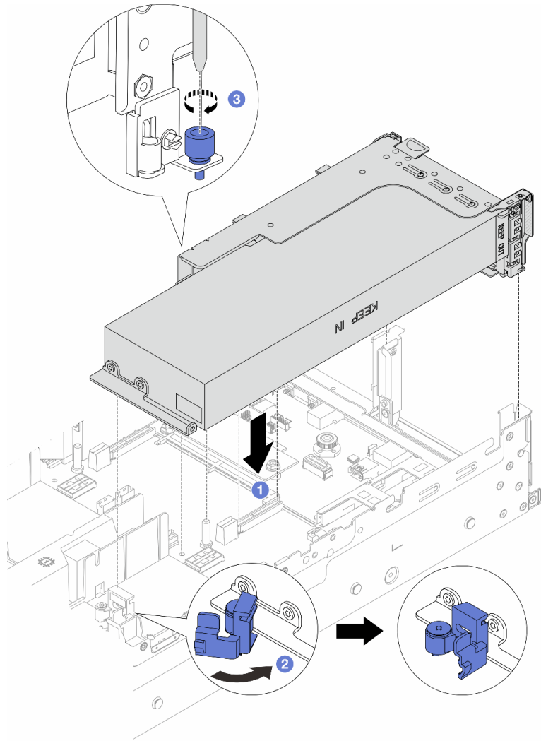
圖例 93. 安裝配備 GPU 配接卡的擴充卡 1 組件
