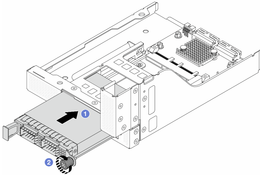
圖例 57. 安裝 OCP 模組
