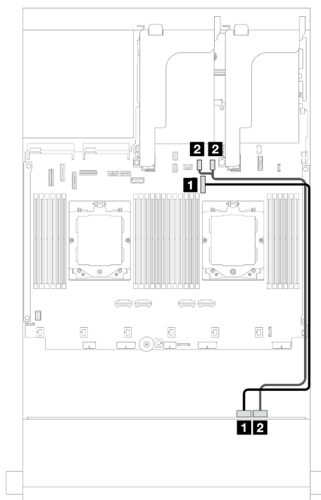
圖例 576. NVMe 纜線佈線
