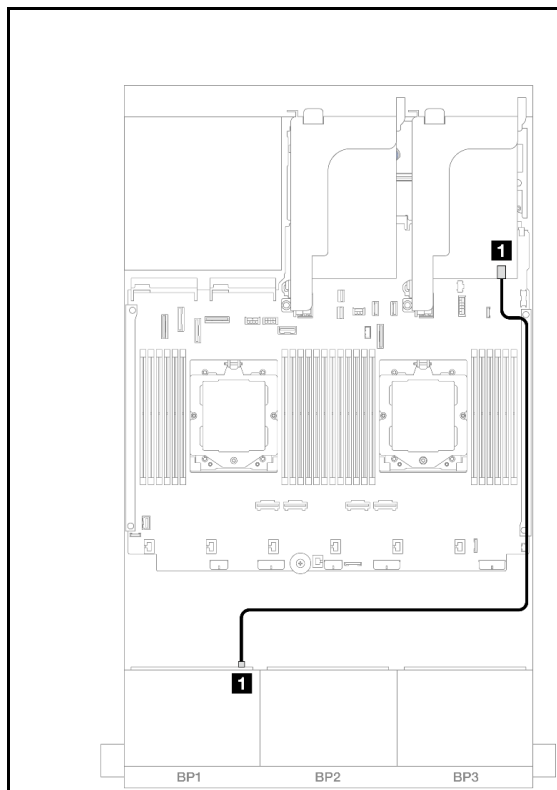
圖例 431. SAS/SATA 纜線佈線
