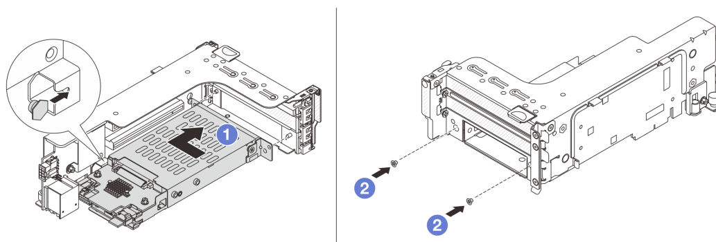
圖例 240. 將 7 公釐框架安裝到擴充卡組件
