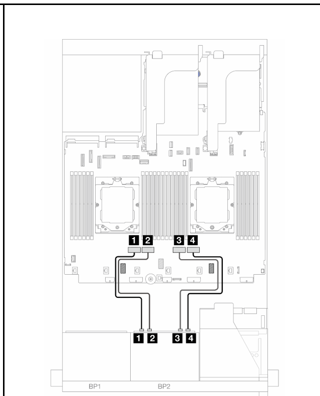
圖例 417. NVMe 纜線佈線
