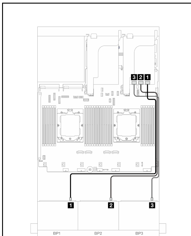
圖例 440. 前方背板纜線佈線
