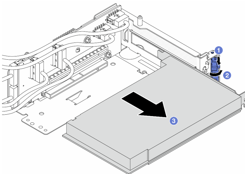
圖例 64. 從擴充卡 5 匣卸下 PCIe 配接卡
