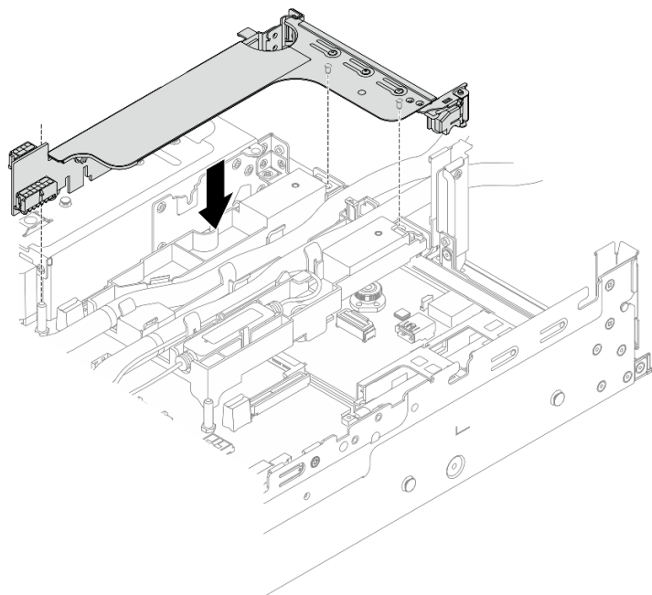
圖例 112. 安裝 1FH 擴充卡匣
