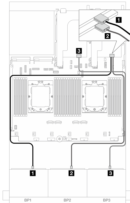
圖例 489. SAS/SATA 纜線佈線至 8i 三模式配接卡
