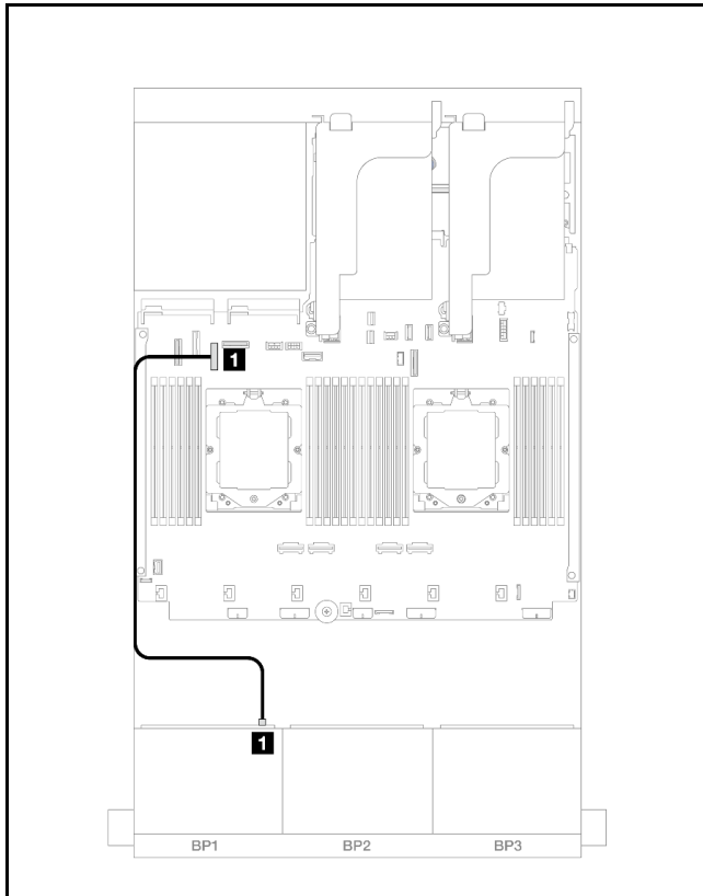
圖例 360. 安裝了兩個處理器的纜線佈線
