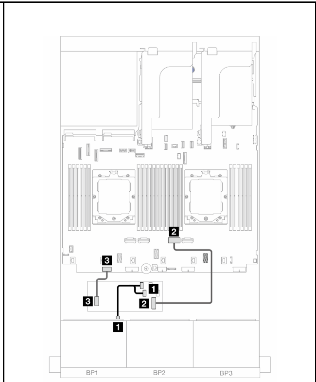
圖例 364. 安裝了一個處理器的纜線佈線
