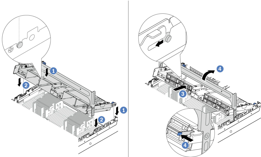
圖例 188. 安裝中間框架和硬碟
