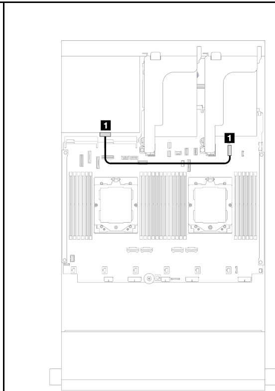
圖例 554. 後方背板電源線佈線
