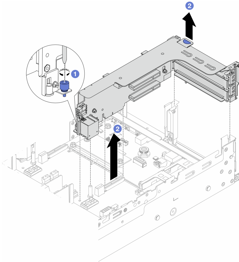
圖例 264. 卸下擴充卡 1 組件
