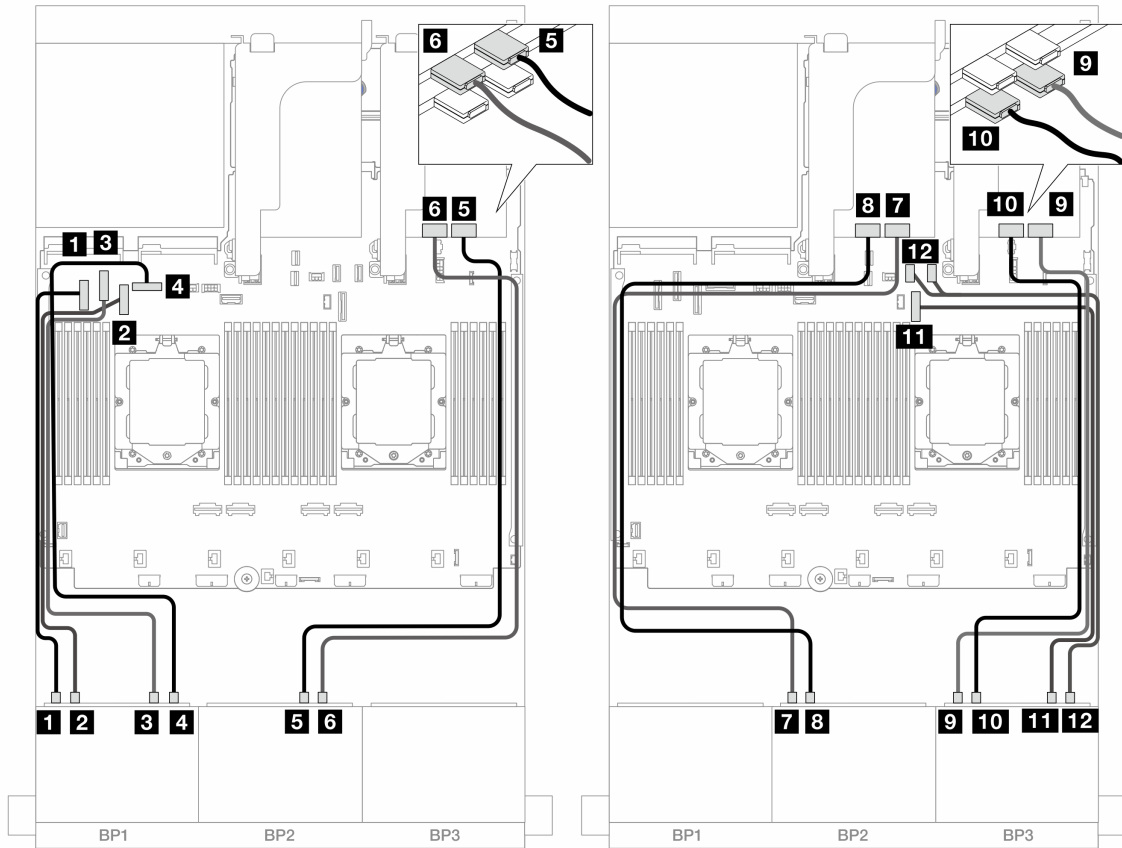
圖例 498. NVMe 纜線佈線至機載接頭和重定時器卡
