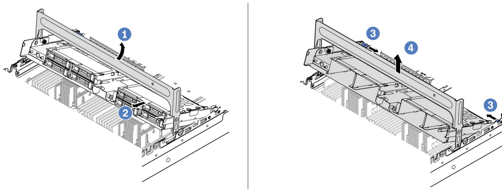
圖例 183. 卸下中間框架
