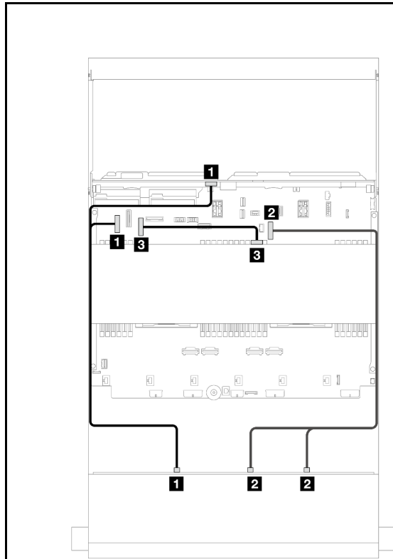
圖例 563. 前方/中間/後方背板信號線佈線
