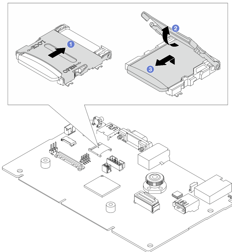
圖例 181. 卸下 MicroSD 卡
