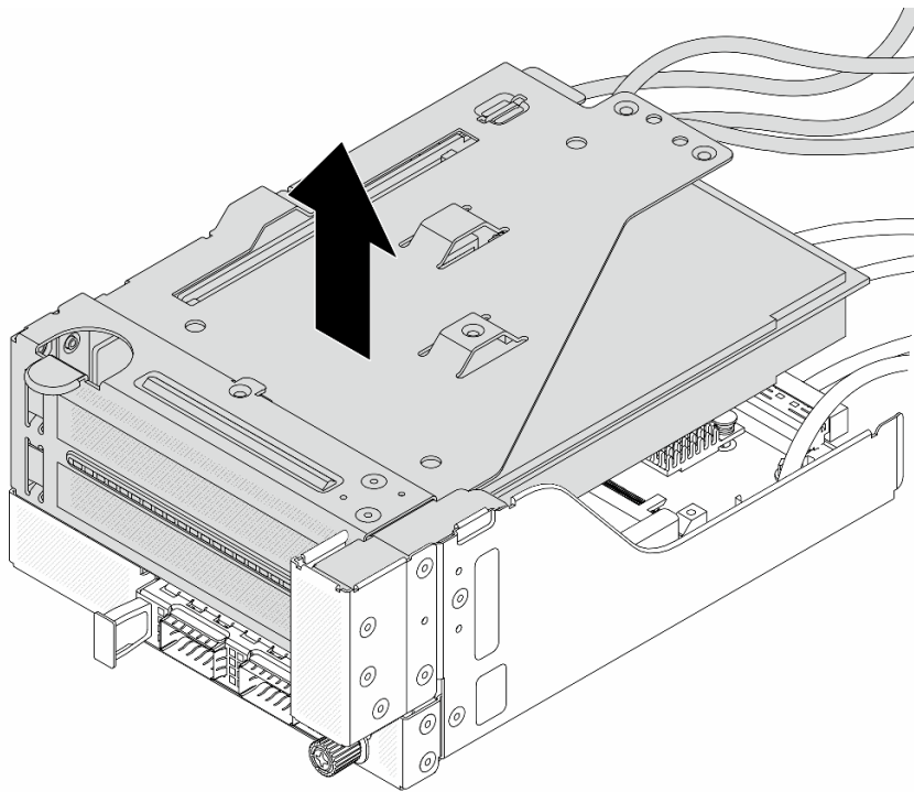
圖例 63. 抬起擴充卡 5 組件
