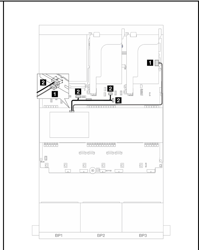
圖例 470. 中間背板纜線佈線
