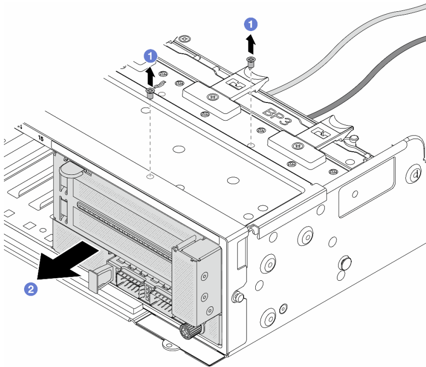
圖例 52. 卸下前配接器組件
