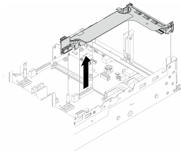
圖例 303. 卸下擴充卡托架
