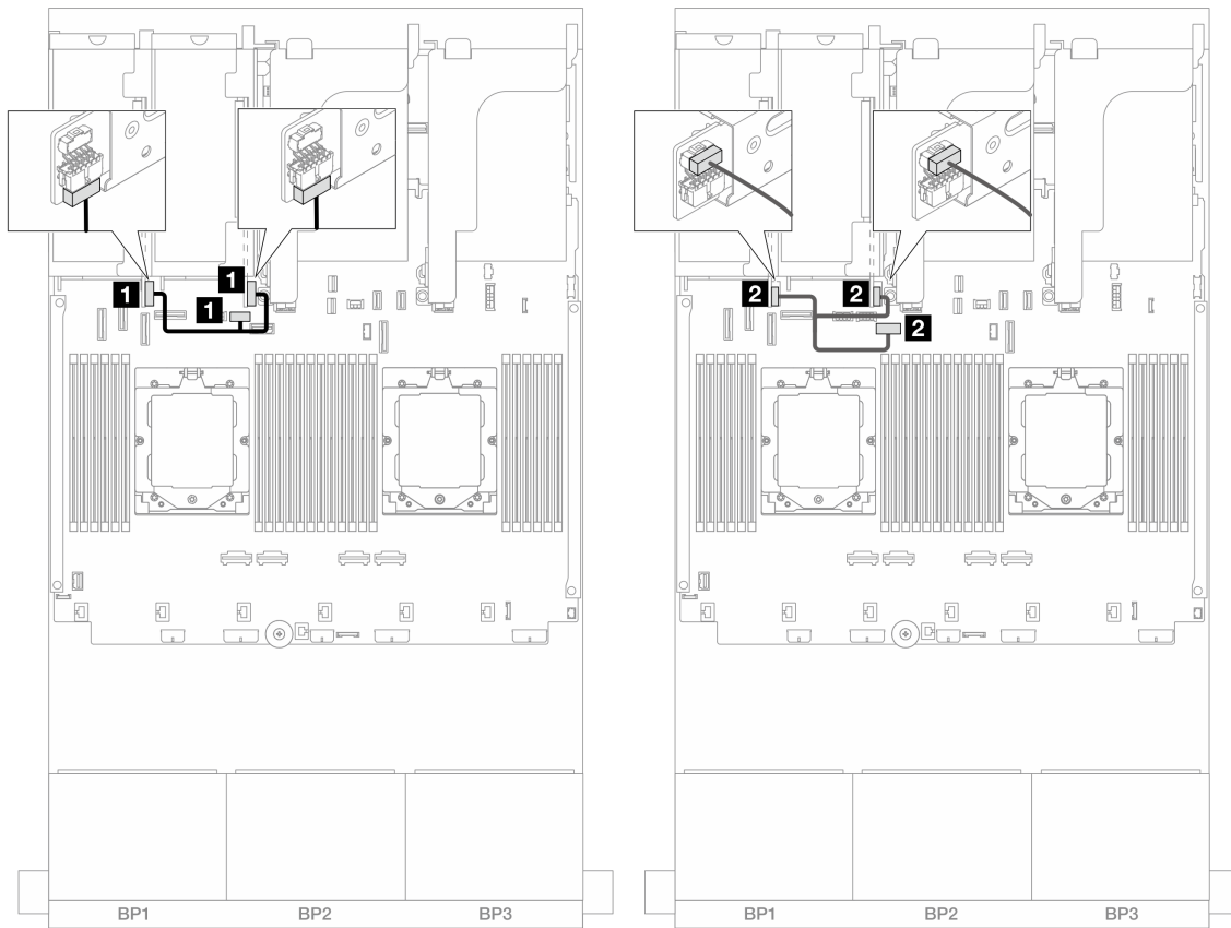
圖例 353. 擴充卡 3/4 電源及側頻纜線佈線
