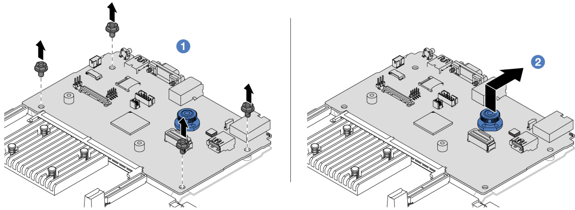
圖例 293. 將系統 I/O 板與處理器板分開
