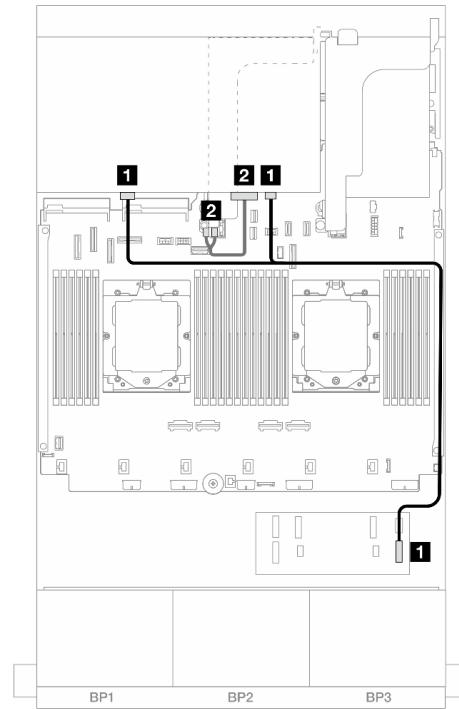
圖例 465. 後方背板纜線佈線
