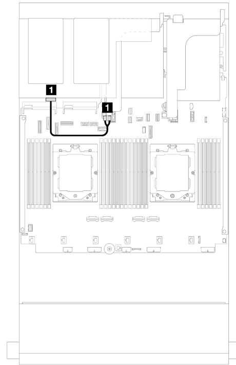
圖例 581. 後方背板電源線佈線
