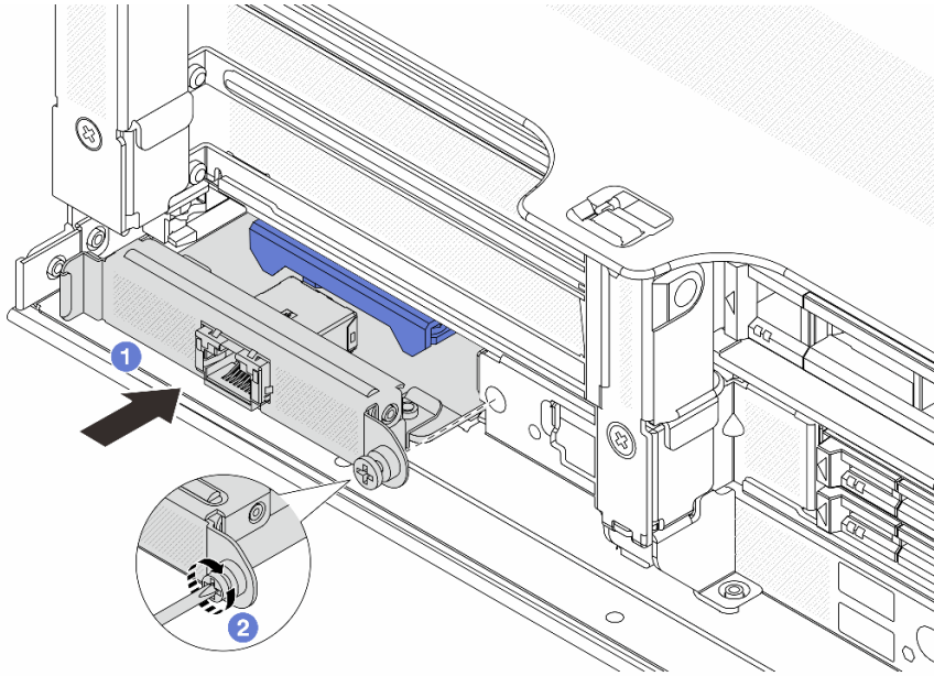
圖例 131. 安裝管理 NIC 配接卡
