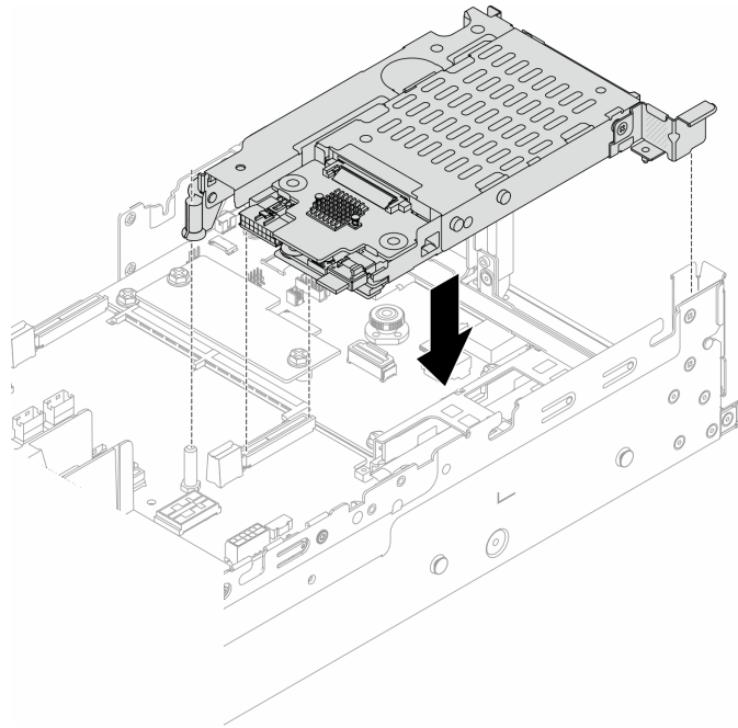
圖例 242. 安裝 7 公釐 SSD 擴充卡匣
