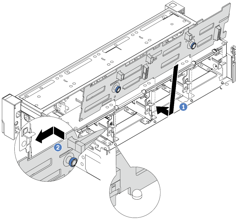
圖例 76. 安裝 3.5 吋硬碟背板
