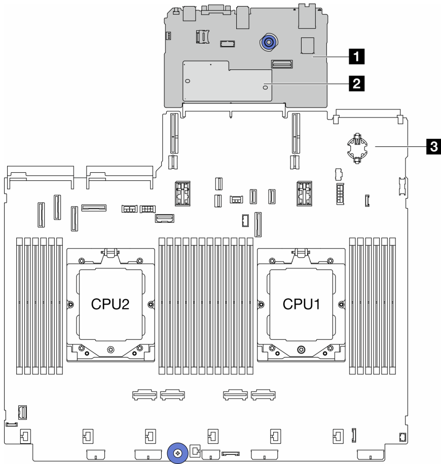
圖例 289. 主機板組件佈置
