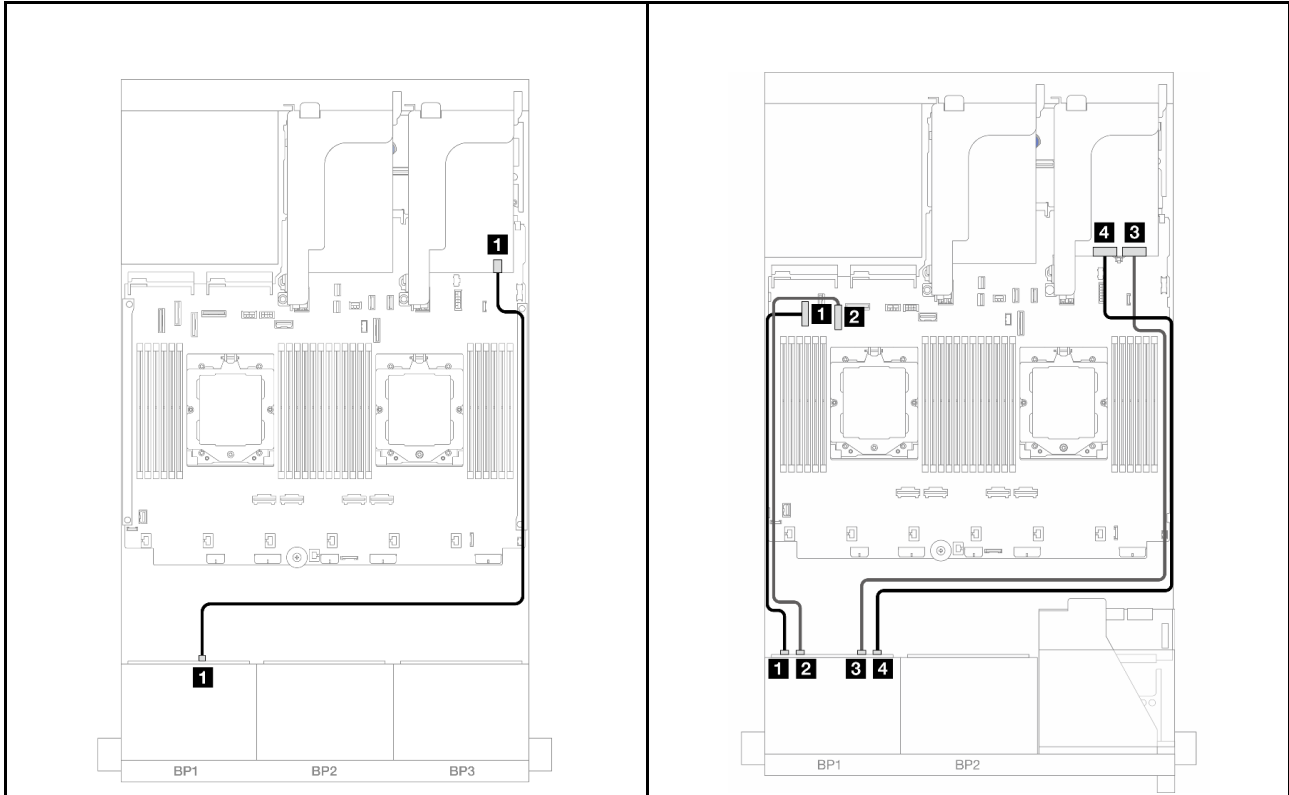
圖例 372. SAS/SATA 纜線佈線
