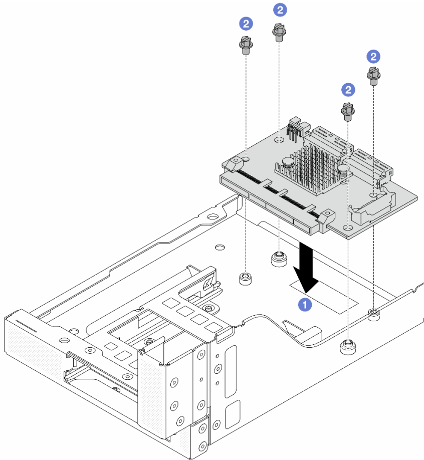
圖例 56. 安裝正面 OCP 轉插卡
