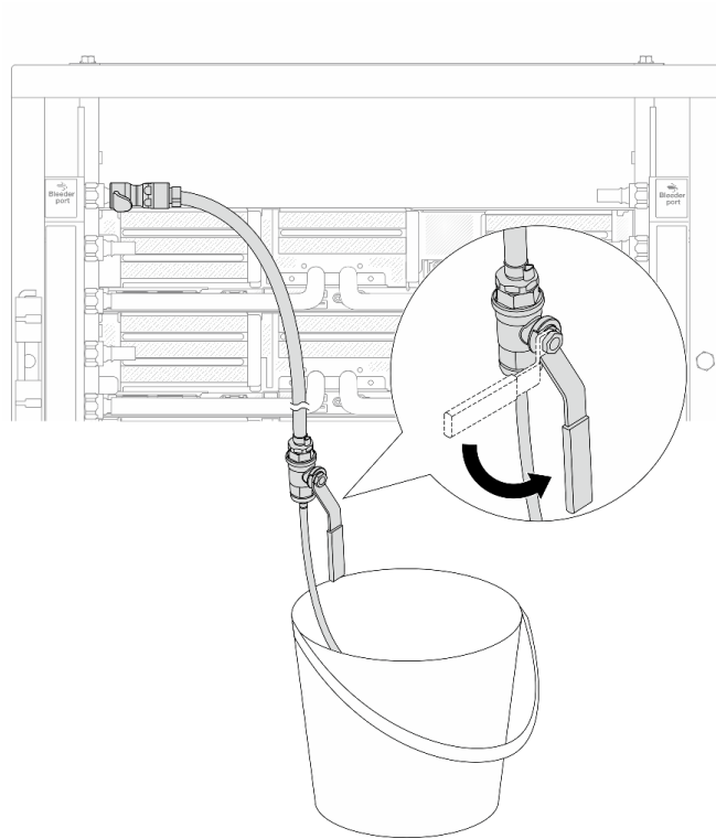
圖例 173. 開啟供應側的洩放閥門
