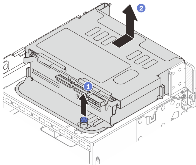
圖例 243. 卸下 4 x 2.5 吋背面框架
