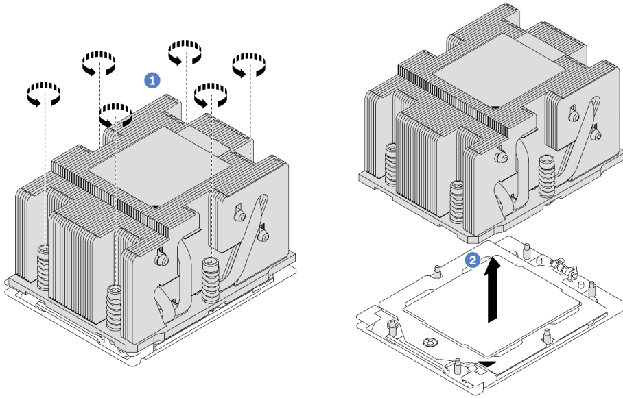
圖例 194. 卸下標準散熱槽
