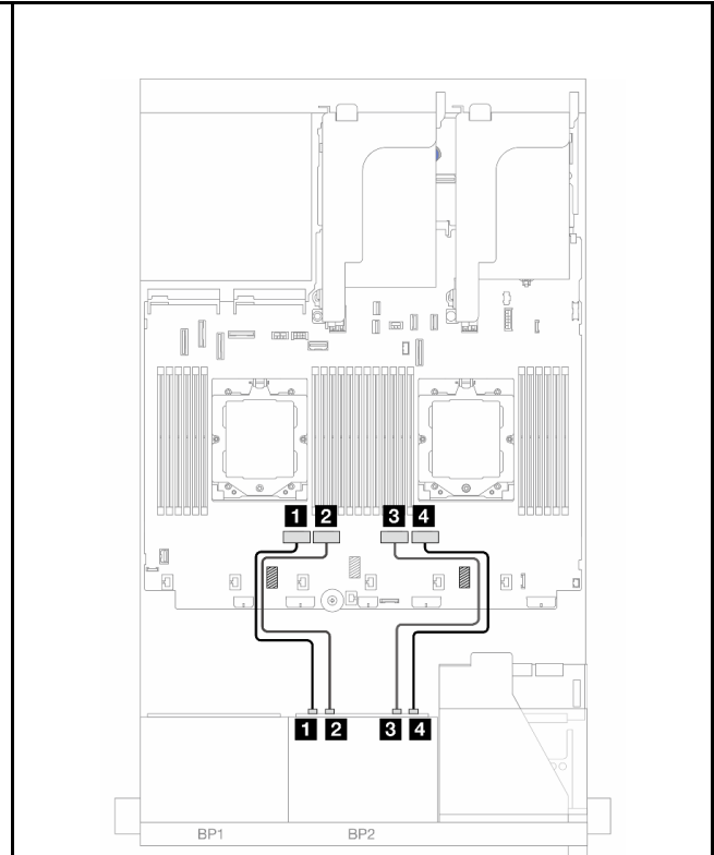
圖例 415. NVMe 纜線佈線
