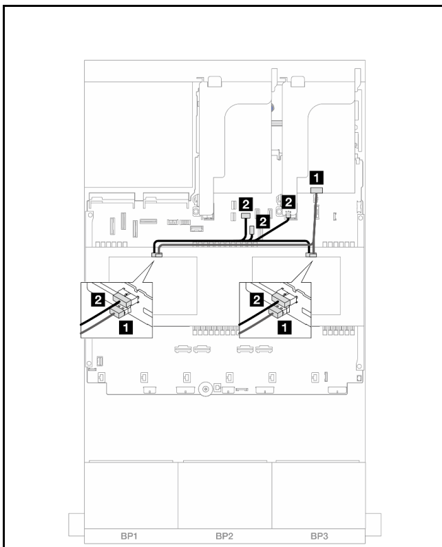
圖例 400. 中間背板纜線佈線
