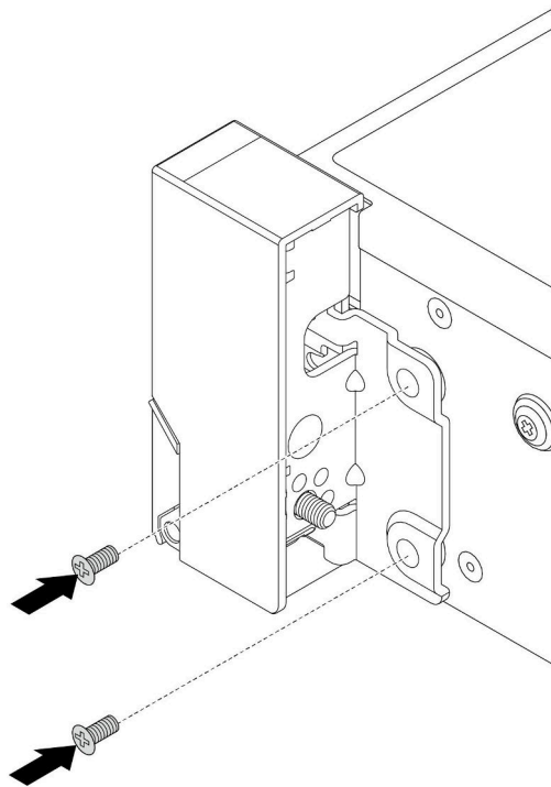
圖例 208. 鎖上螺絲
