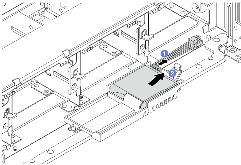
圖例 214. 從超級電容固定器卸下 RAID 快閃記憶體電源模組
