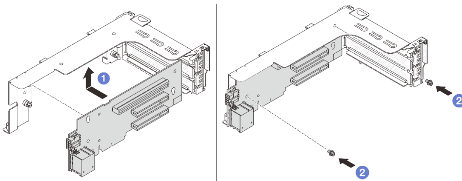
圖例 274. 將擴充卡安裝到擴充卡 1 或 2 匣
