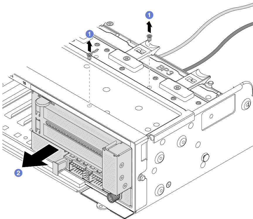
圖例 38. 卸下前配接器組件
