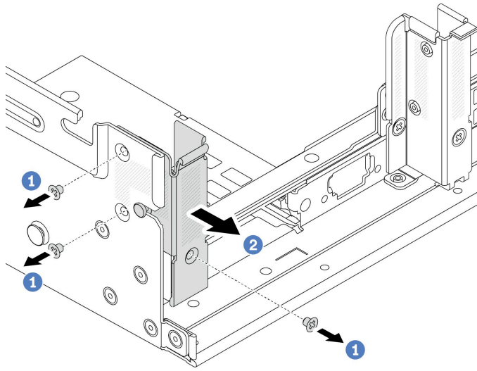
圖例 226. 卸下 A1 後壁托架 (左)
