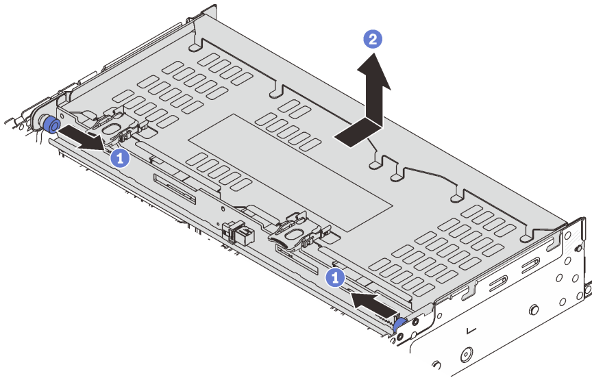
圖例 255. 卸下 4 x 3.5 吋背面框架
