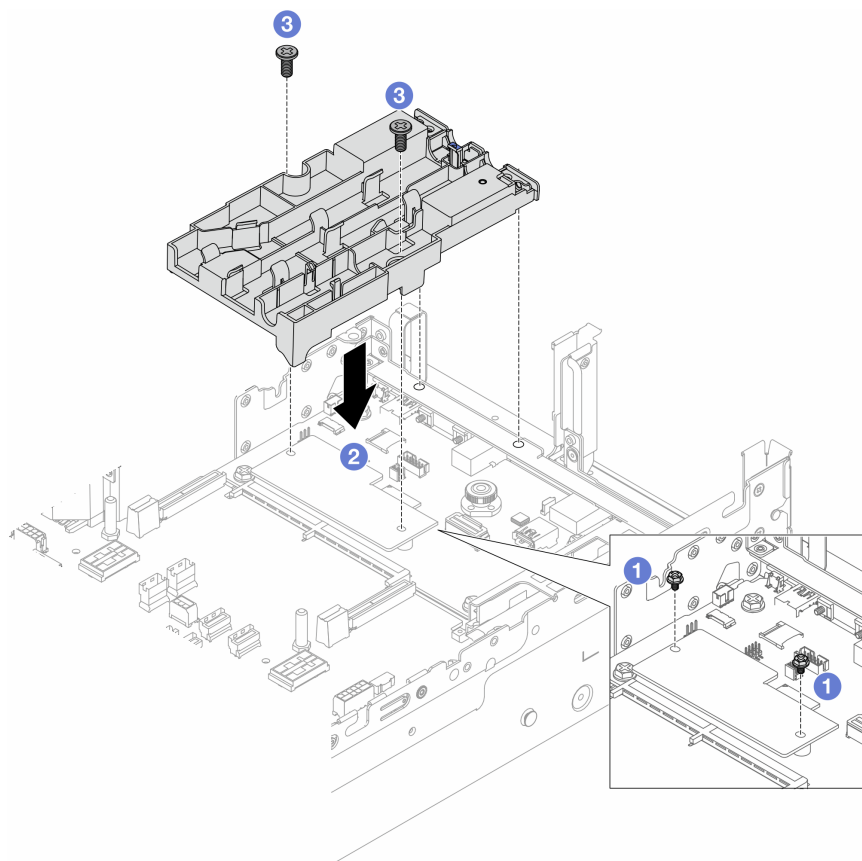
圖例 106. 安裝水管固定器
