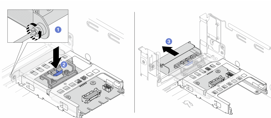
圖例 60. 卸下背面 OCP 轉插卡
