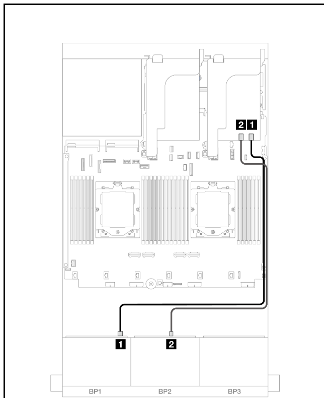
圖例 416. SAS/SATA 纜線佈線
