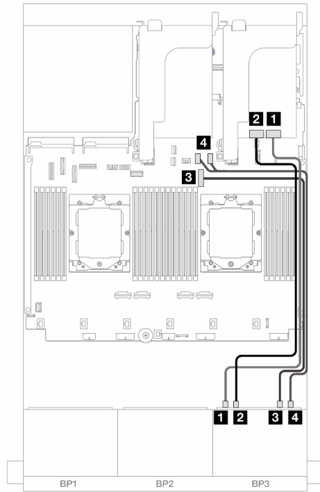
圖例 511. NVMe 纜線佈線
