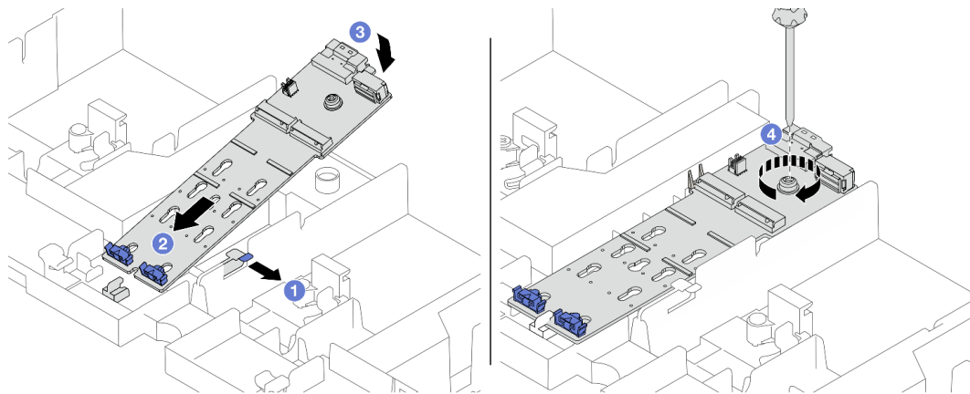
圖例 124. 將 M.2 背板安裝在空氣擋板上
