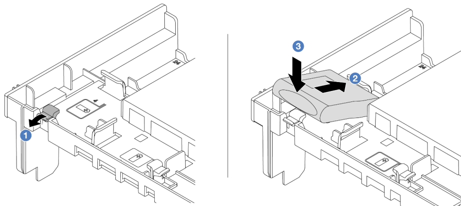
圖例 219. 將 RAID 快閃記憶體電源模組安裝在空氣擋板上
