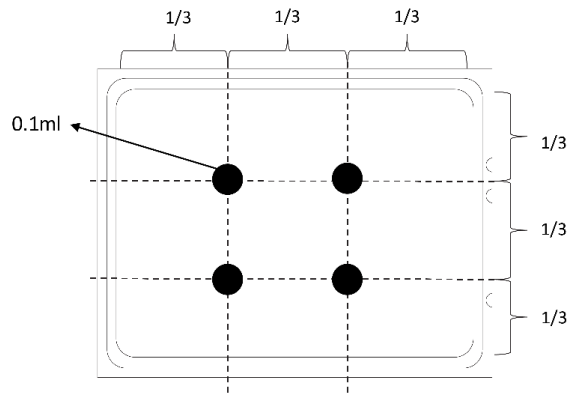
圖例 200. 塗上散熱膏
