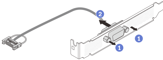
圖例 305. 拆卸序列埠模組
