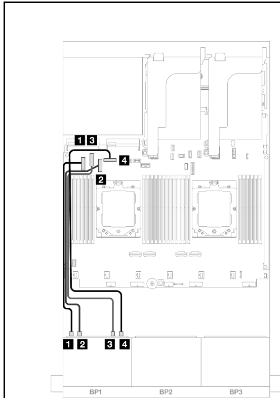
圖例 384. 安裝了兩個處理器的纜線佈線
