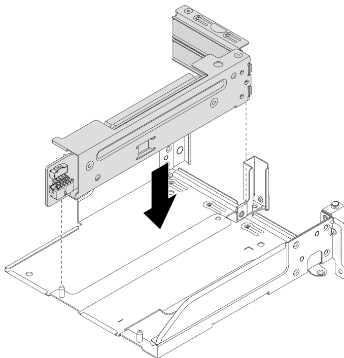
圖例 283. 安裝擴充卡 3/4 組件
