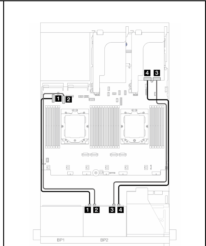
圖例 419. NVMe 纜線佈線
