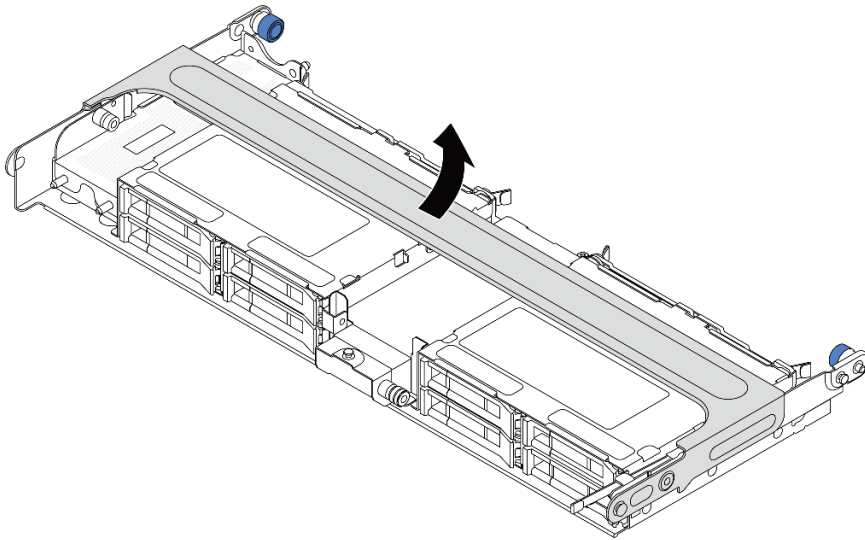
圖例 221. 打開中間框架的把手
