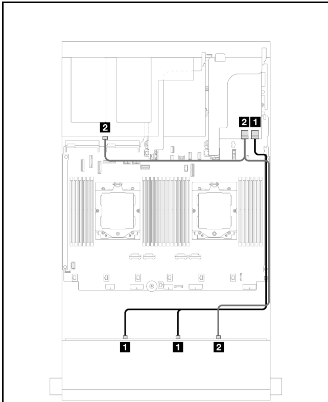
圖例 551. 前方/後方背板信號線佈線
