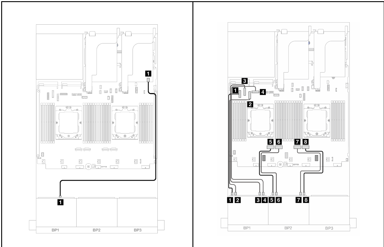
圖例 433. SAS/SATA 纜線佈線
