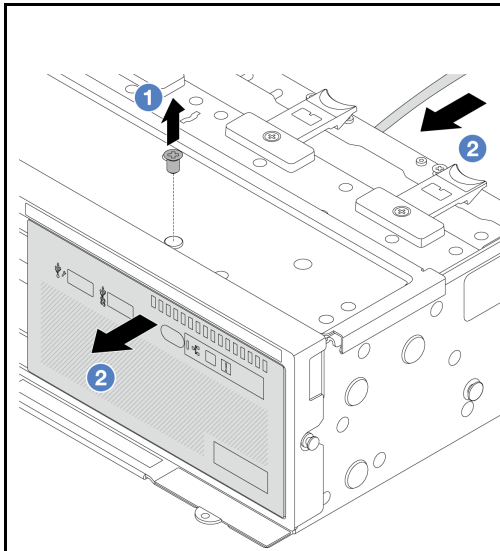
圖例 78. 具有前方操作面板的正面 I/O 模組
