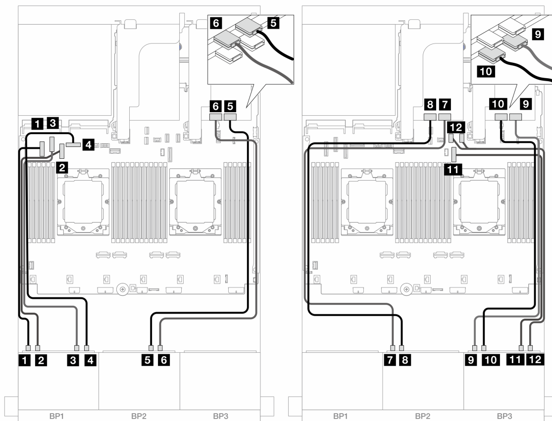
圖例 492. NVMe 纜線佈線至機載接頭和重定時器卡
