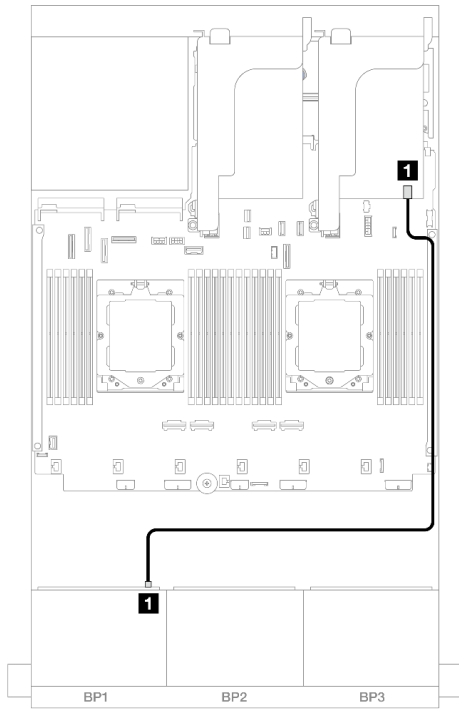
圖例 429. SAS/SATA 纜線佈線
