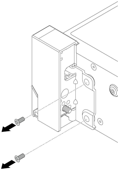
圖例 205. 卸下螺絲
