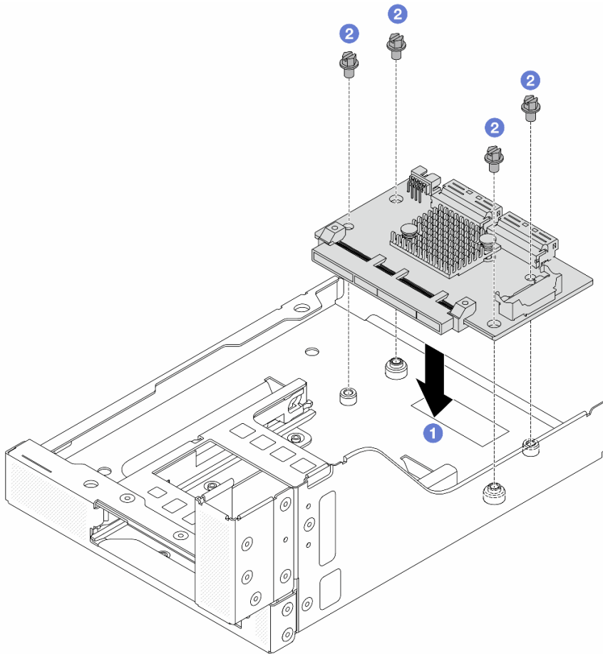
圖例 44. 安裝正面 OCP 轉插卡
