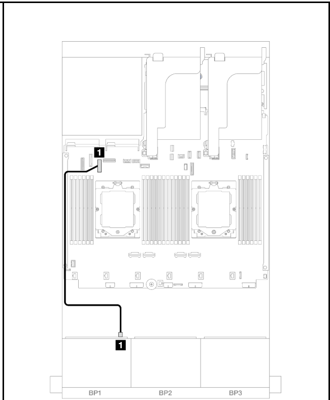
圖例 383. NVMe 纜線佈線
