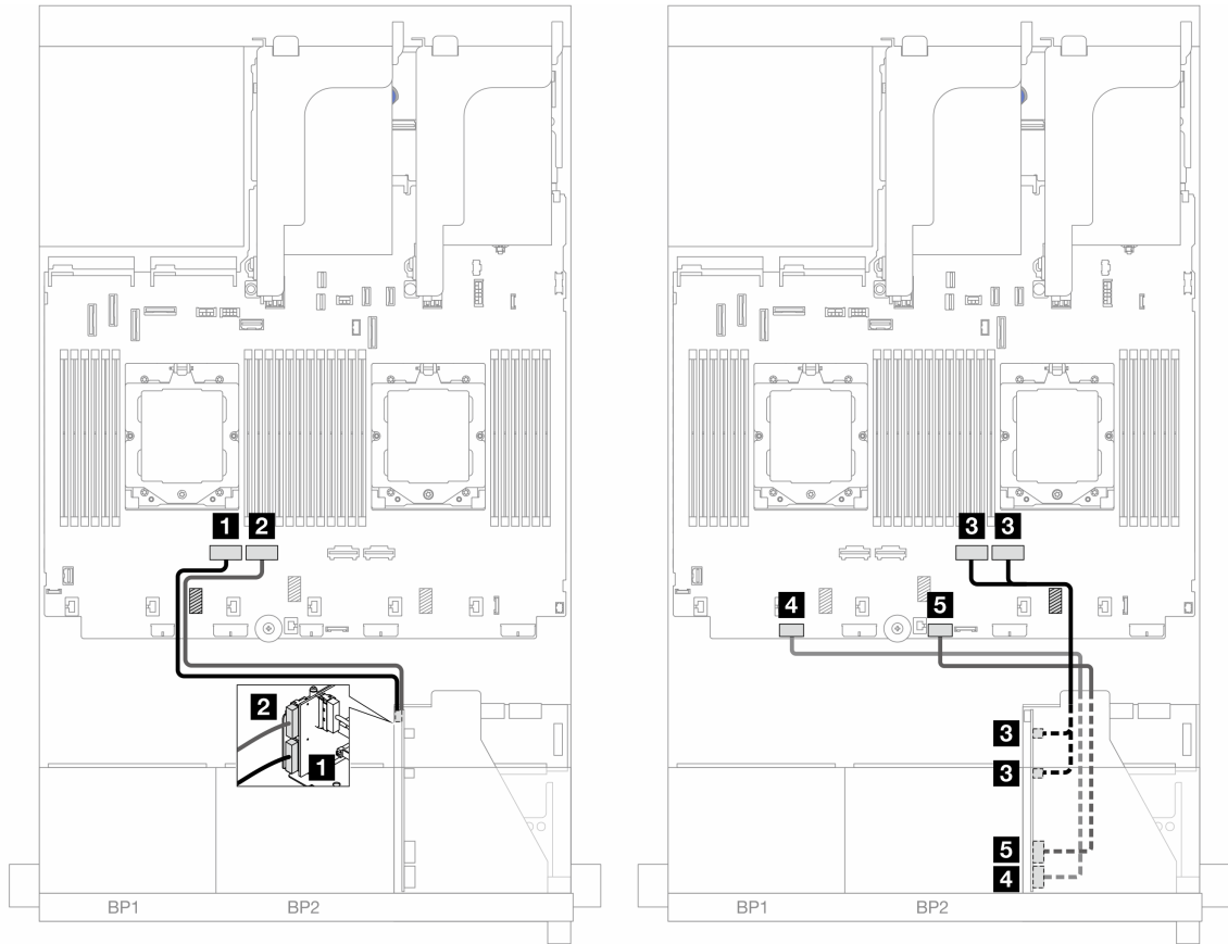
圖例 356. 含擴充卡 3/4 的配置的纜線佈線
