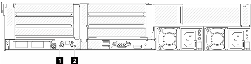
圖例 591. 背面系統 LED
