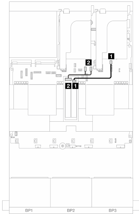
圖例 335. SATA/NVMe 纜線佈線
