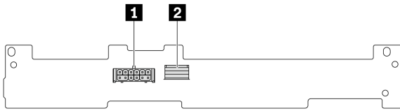
圖例 321. 2 x 3.5 吋 SAS/SATA 背板接頭
