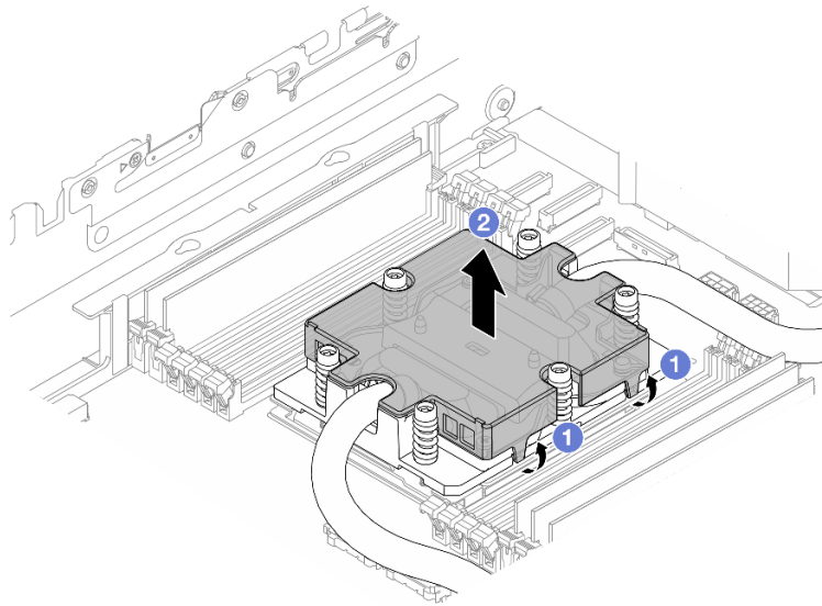
圖例 598. 拆下水冷板蓋
