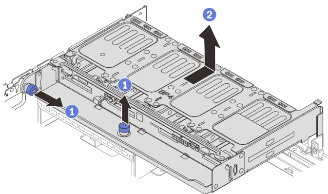
圖例 247. 卸下 8 x 2.5 吋背面框架
