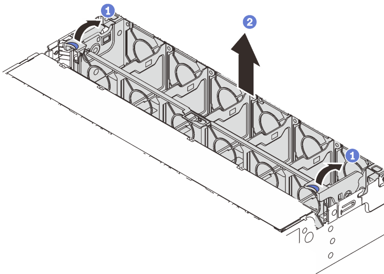
圖例 300. 卸下系統風扇機盒
