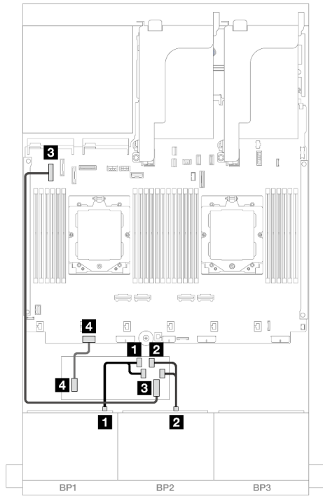
圖例 412. SAS/SATA 纜線佈線
