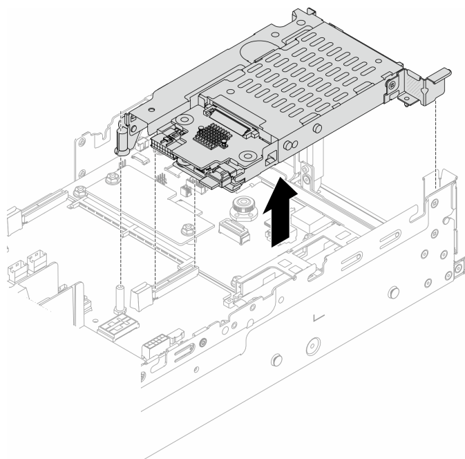
圖例 233. 卸下 7 公釐 SSD 擴充卡匣
