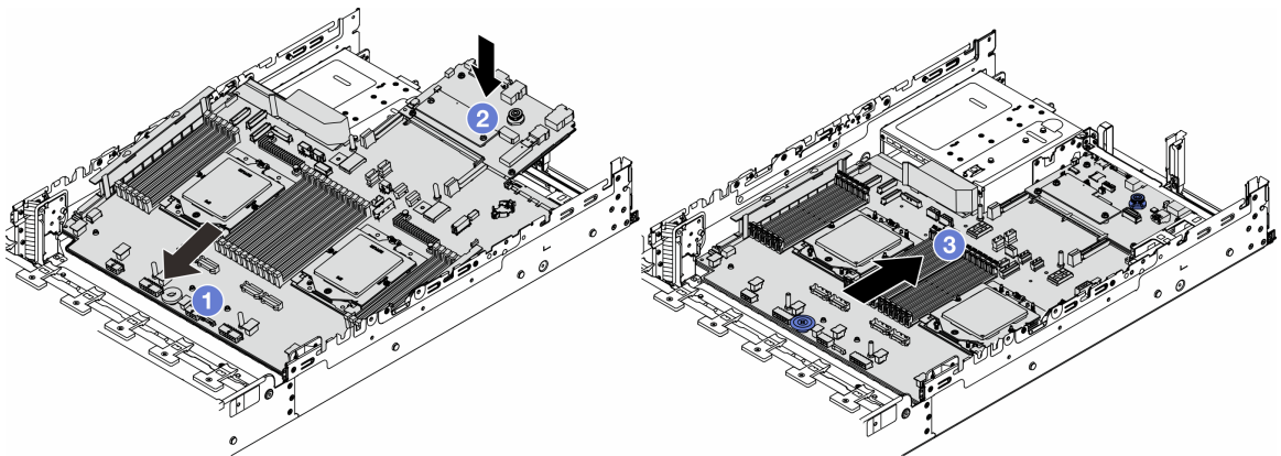
圖例 297. 安裝主機板組件
