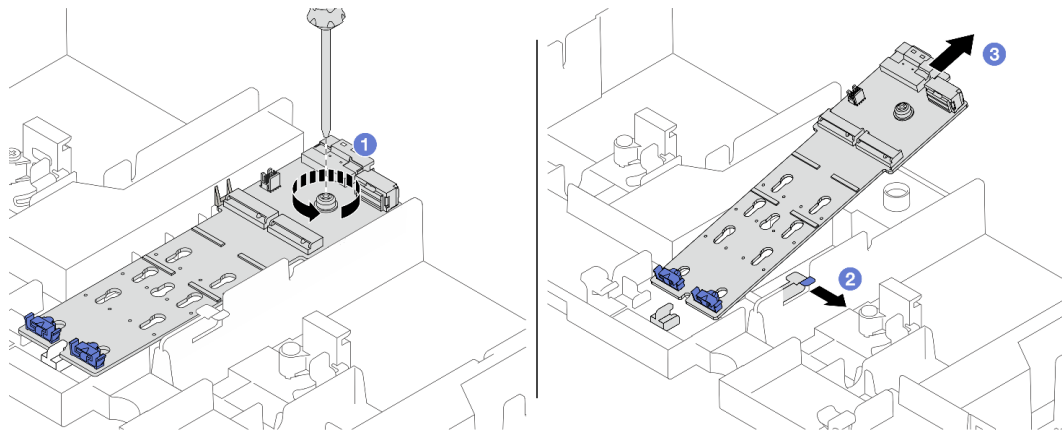
圖例 121. 從空氣擋板卸下 M.2 背板
