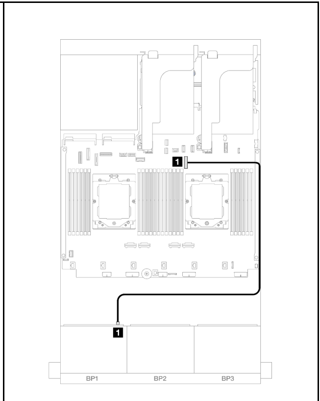
圖例 361. 安裝了一個處理器的纜線佈線
