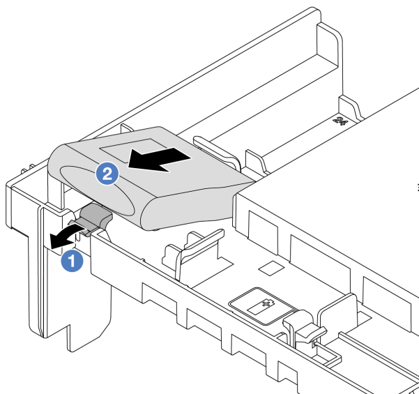
圖例 218. 從空氣擋板卸下 RAID 快閃記憶體電源模組
