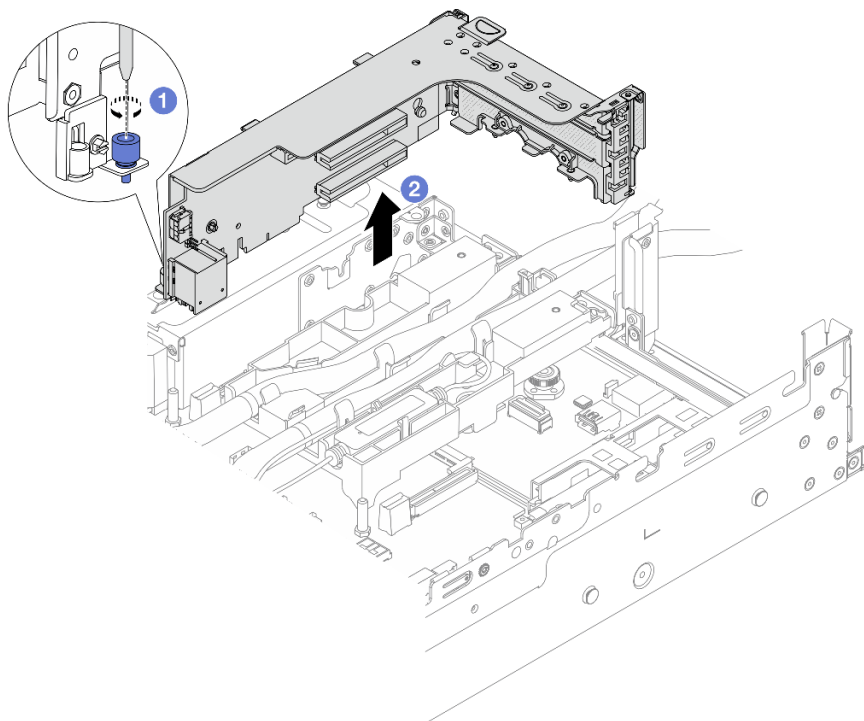
圖例 102. 卸下 3FH 擴充卡匣
