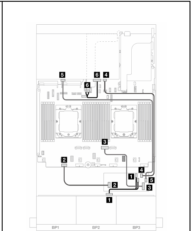
圖例 539. 安裝了一個處理器的纜線佈線
