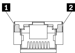
圖例 592. XCC 系統管理埠 LED
