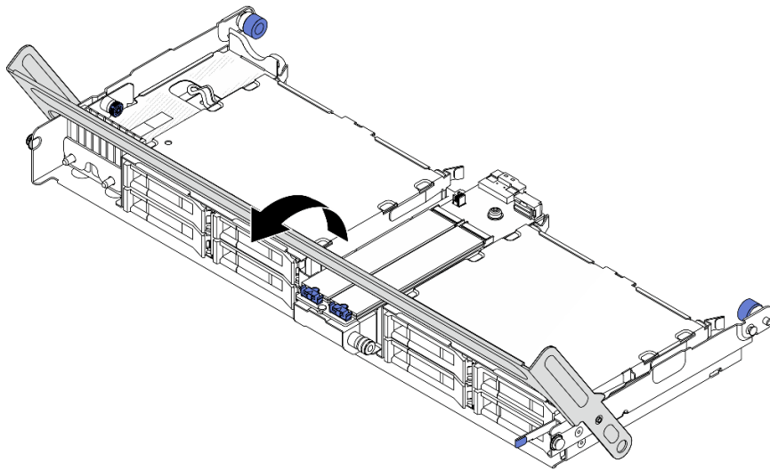
圖例 122. 打開中間框架的把手
