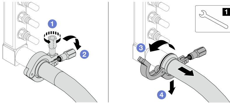
圖例 146. 將歧管與連接套組分開
