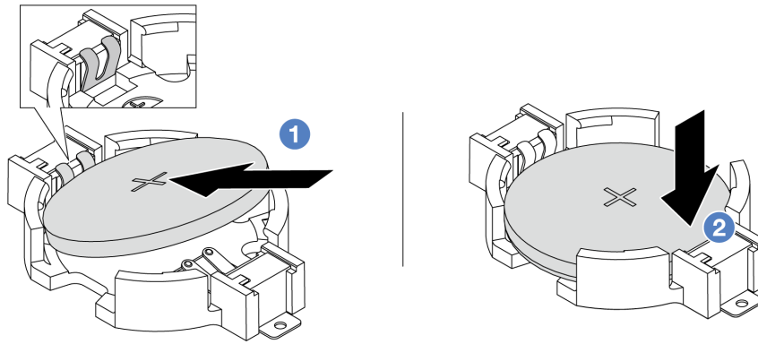
圖例 37. 安裝 CMOS 電池
