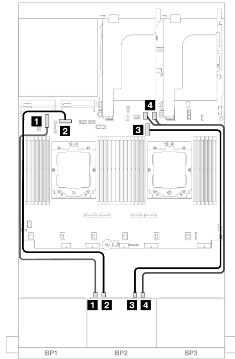
圖例 413. NVMe 纜線佈線
