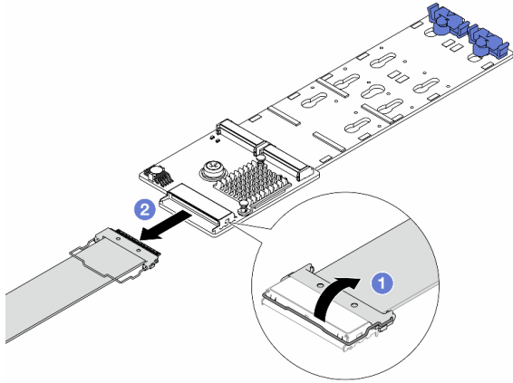
圖例 120. 從 M.2 RAID SATA/NVME 2 機槽背板拔掉纜線
