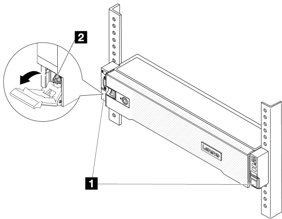
圖例 20. 使伺服器脫離機架
