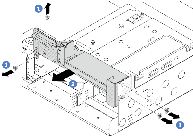
圖例 228. 卸下 C1 後壁托架 (右)
