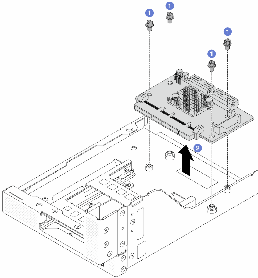
圖例 43. 卸下正面 OCP 轉插卡
