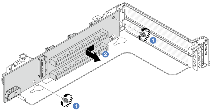
圖例 272. 從擴充卡 3 匣卸下擴充卡
