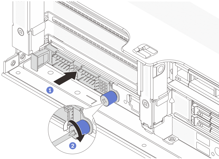
圖例 261. 安裝背面 OCP 模組
