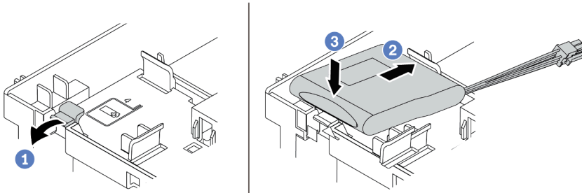
Figura 166. Instalação do módulo de supercapacitor no defletor de ar
