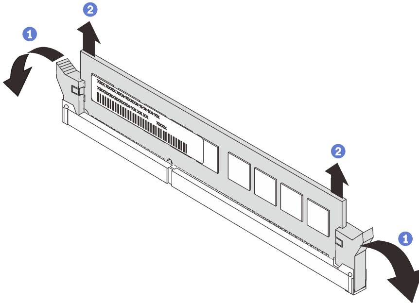
Figura 145. Remoção do módulo de memória
