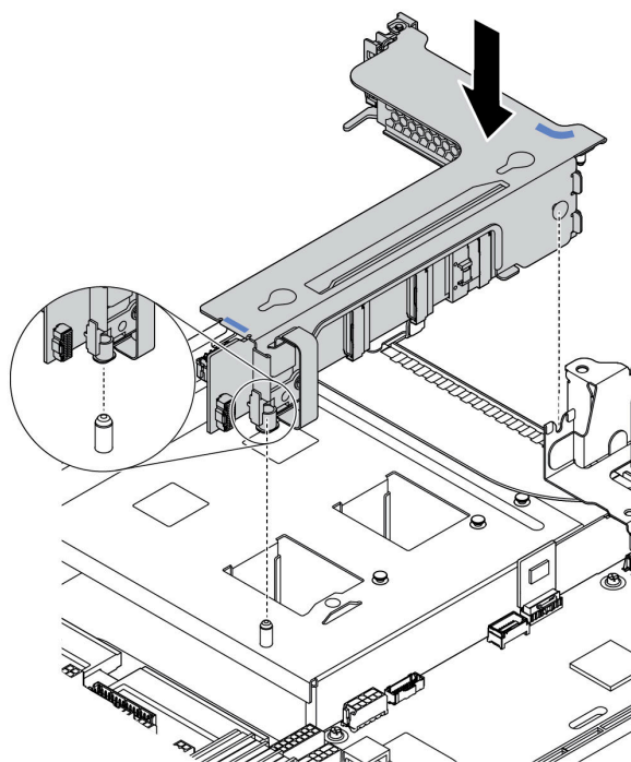
Figura 193. Instalação do conjunto de placa riser 3
