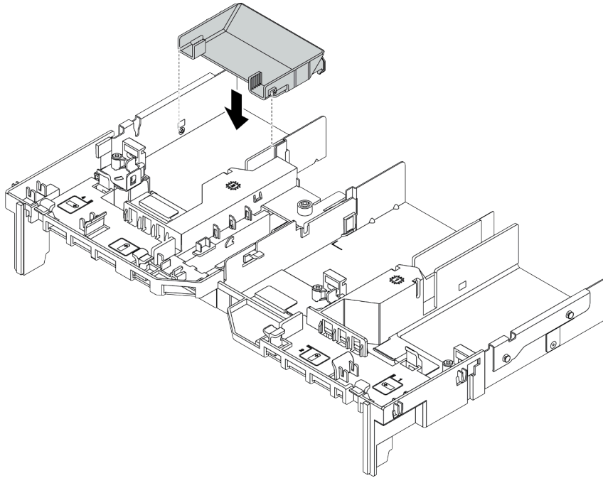
Figura 73. Instalando o defletor de ar do adaptador de GPU complementar
