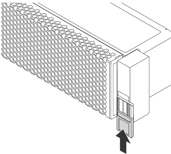
Figura 160. Instalação da placa com etiqueta de identificação
