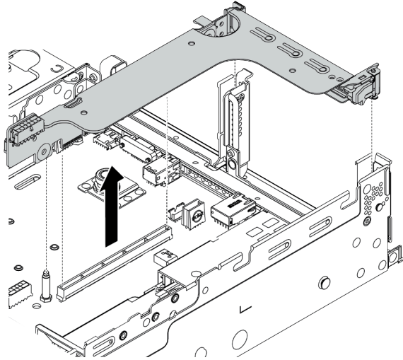
Figura 183. Remoção do conjunto de 1/2 placa riser (suporte para placa riser de um slot)
