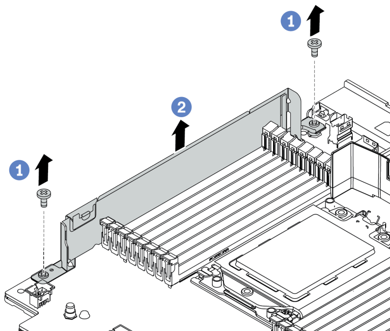
Figura 58. Remoção dos retentores de cabo
