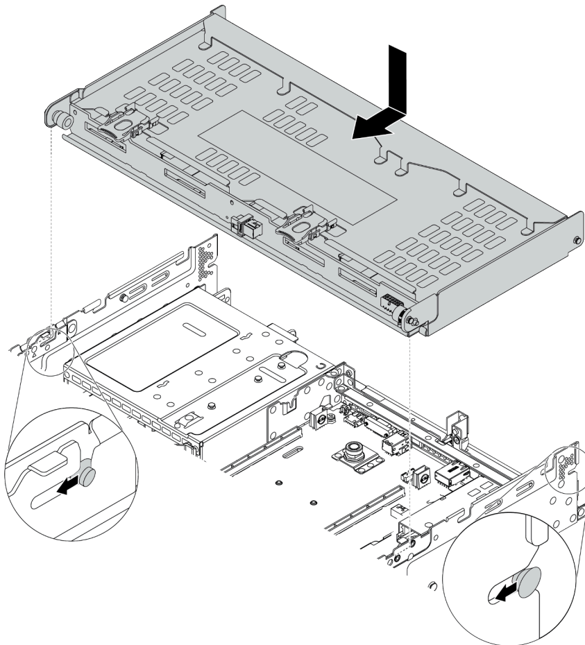
Figura 110. Instalando a gaiola de unidade traseira de 4 x 3,5 polegadas
