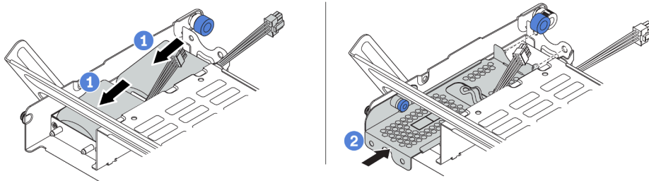
Figura 171. Instalando o módulo de supercapacitor
