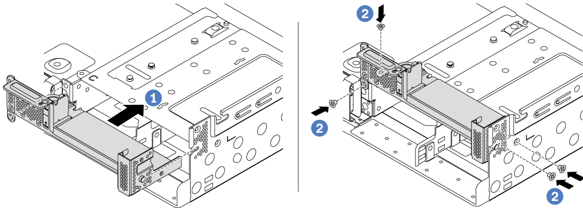
Figura 181. Instalação do suporte de parede traseira C1
