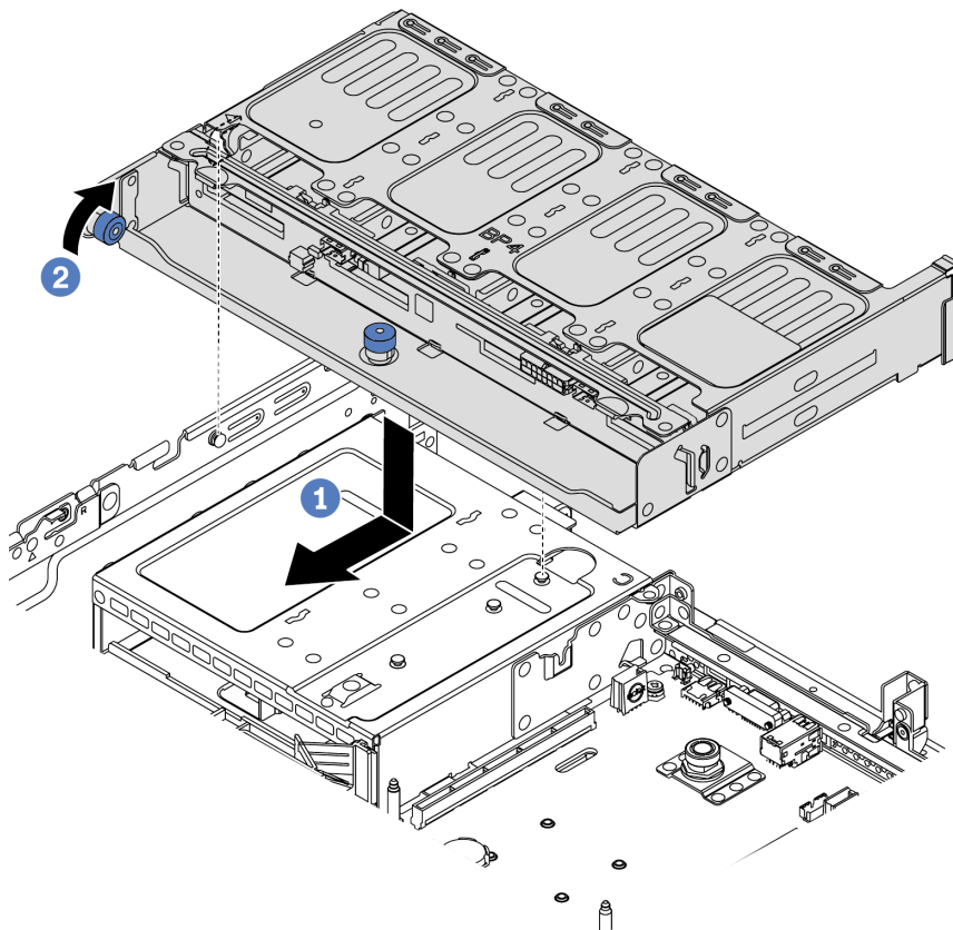
Figura 115. Instalando a gaiola de unidade traseira de 8 x 2,5 polegadas
