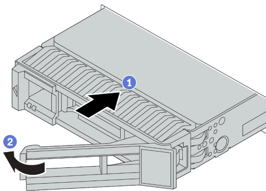
Figura 80. Instalação de unidades hot-swap
