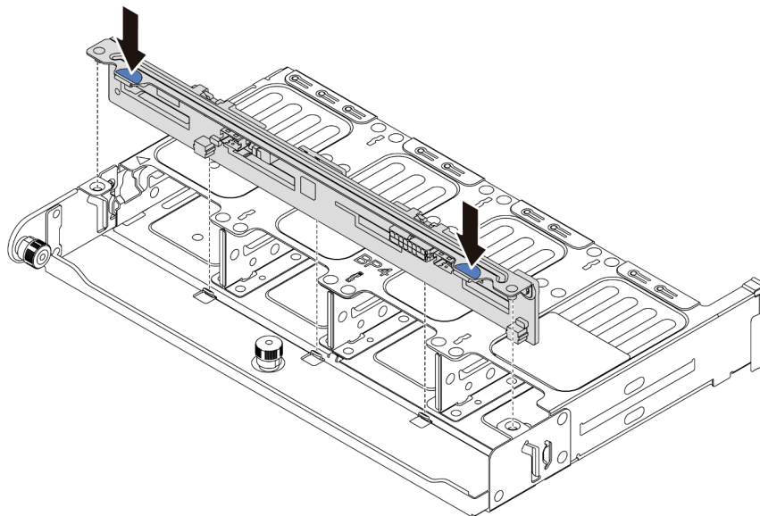
Figura 86. Instalação do painel traseiro da unidade de 8 x 2,5 polegadas
