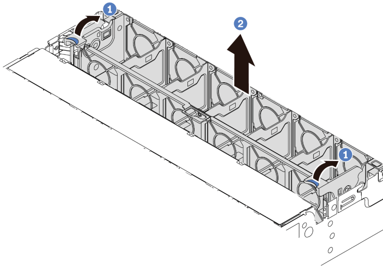
Figura 204. Remoção do compartimento do ventilador do sistema
