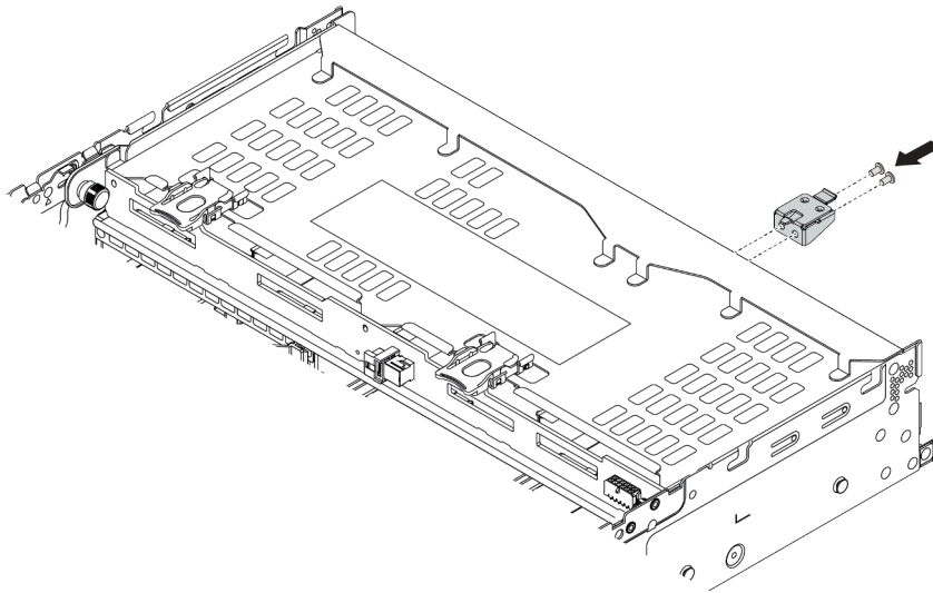
Figura 111. Instalando o suporte de apoio da tampa superior
