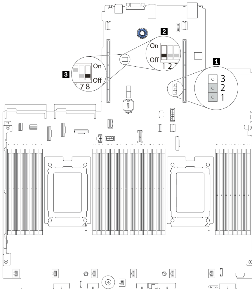
Figura 13. Os locais do bloco de comutador e do jumper na placa-mãe
