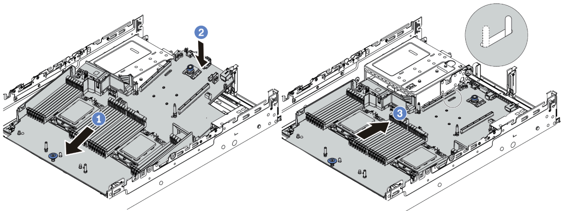
Figura 218. Instalação da placa-mãe
