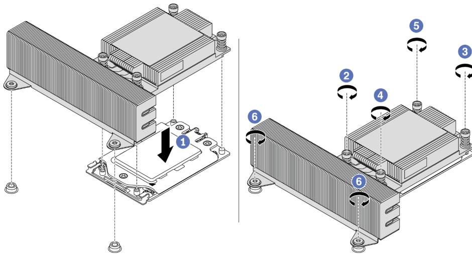
Figura 216. Instalando um dissipador de calor de desempenho
