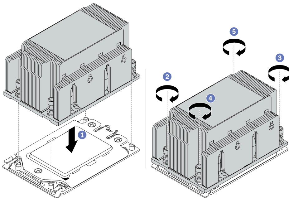
Figura 215. Instalando um dissipador de calor padrão
