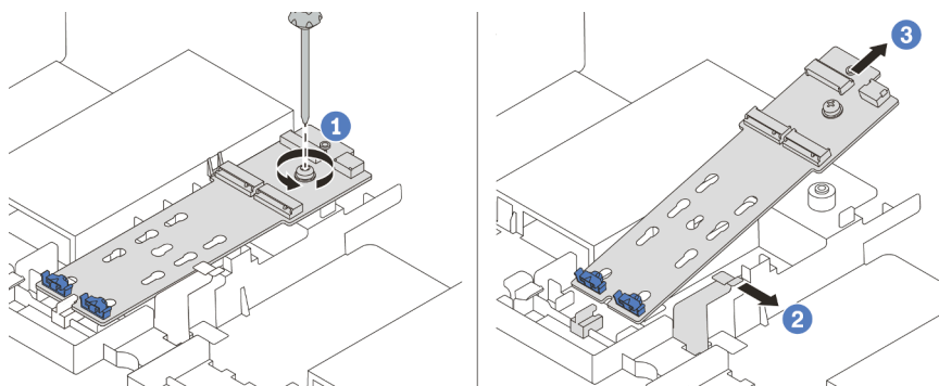
Figura 139. Remoção do adaptador M.2
