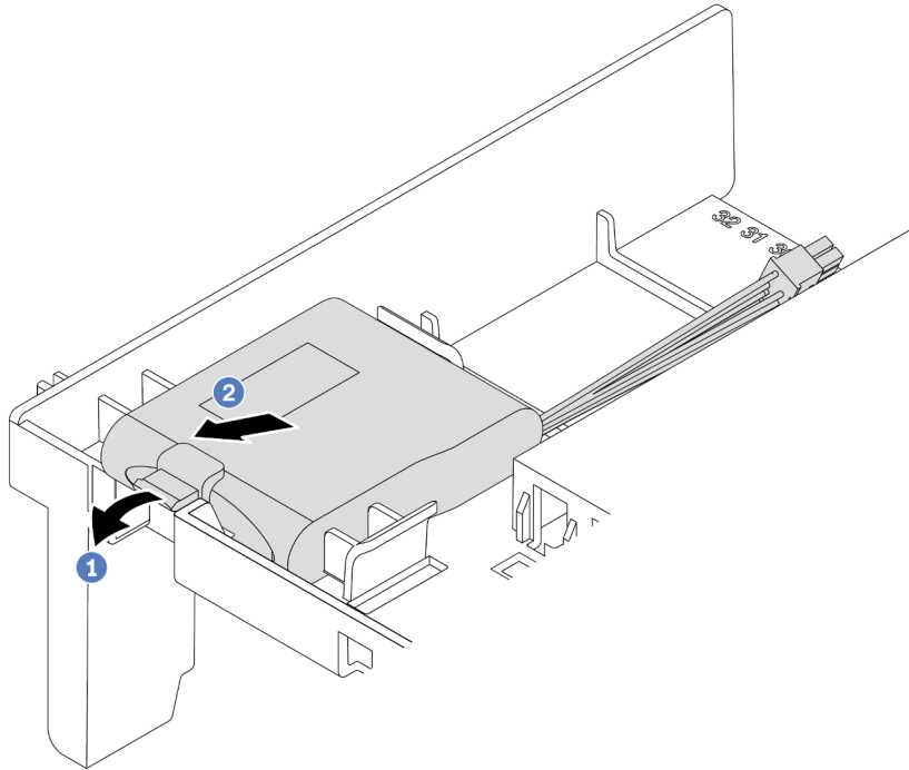
Figura 165. Remoção do módulo de supercapacitor
