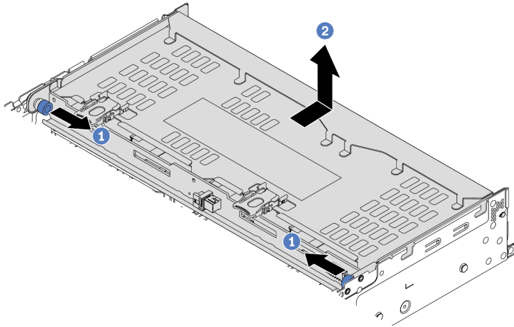
Figura 109. Removendo a gaiola de unidade traseira de 4 x 3,5 pol.
