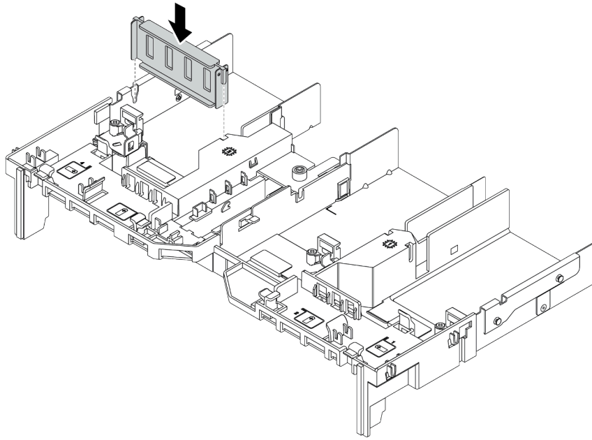
Figura 72. Instalando o preenchimento da GPU
