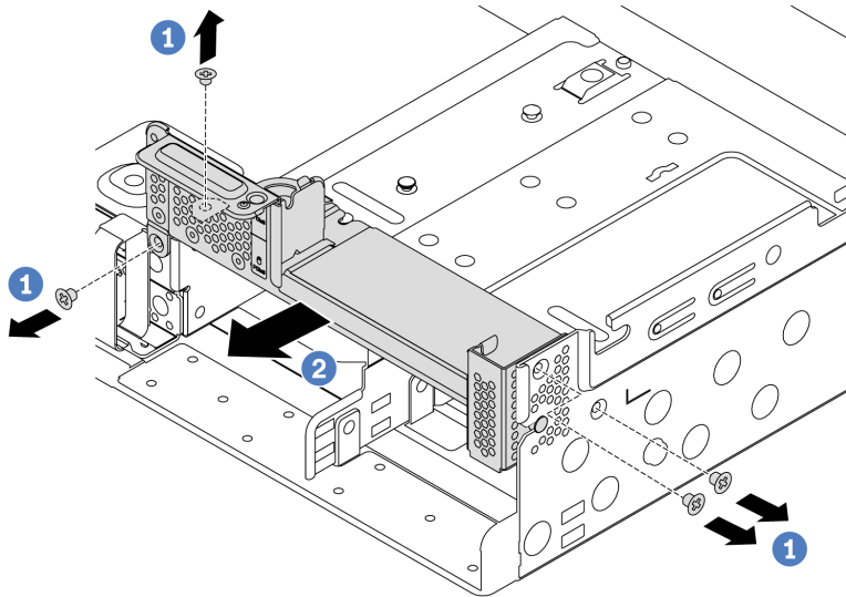
Figura 180. Remoção do suporte de parede traseira C1
