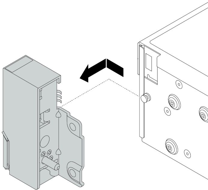
Figura 156. Remoção da trava do rack
