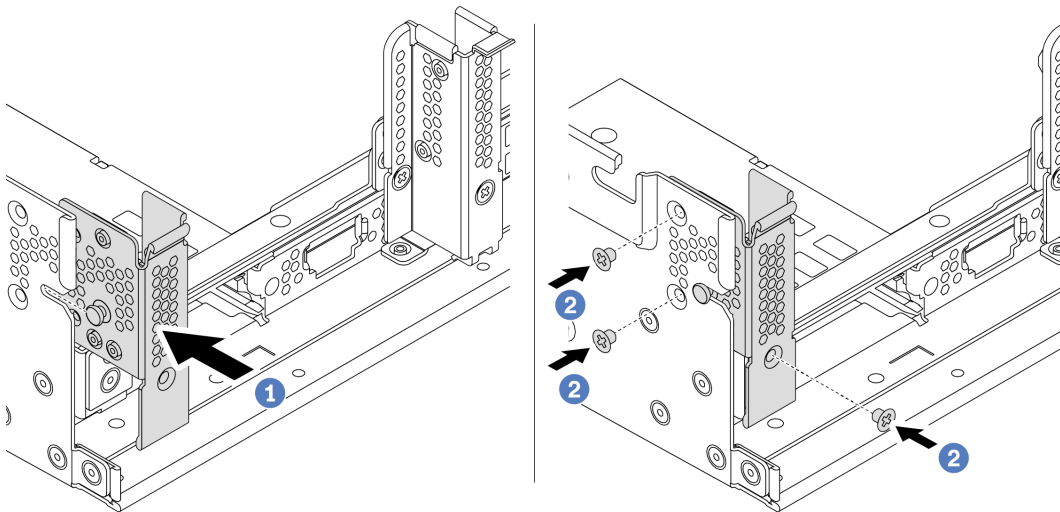
Figura 177. Instalação do suporte de parede traseira A1
