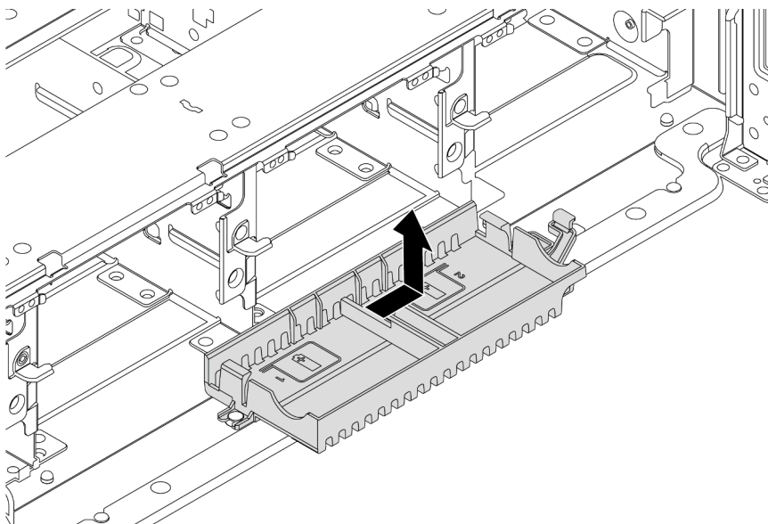
Figura 173. Remoção do suporte de supercapacitor
