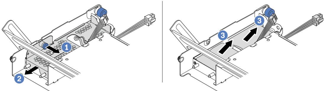
Figura 168. Removendo o módulo de supercapacitor
