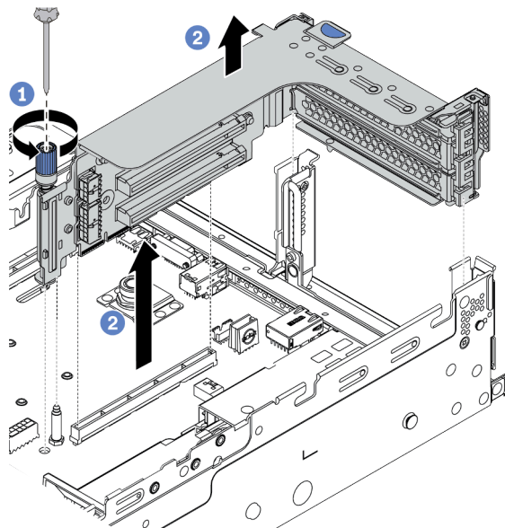
Figura 182. Remoção do conjunto de 1/2 placa riser (suporte de três slots)
