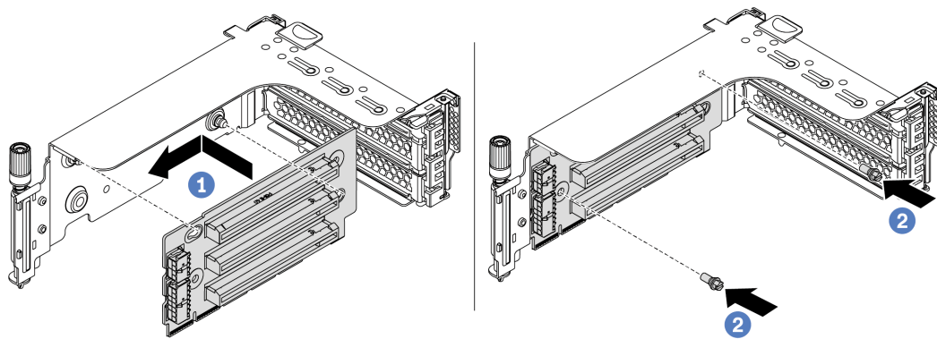
Figura 188. Instalação da placa riser (suporte para placa riser de três slots)
