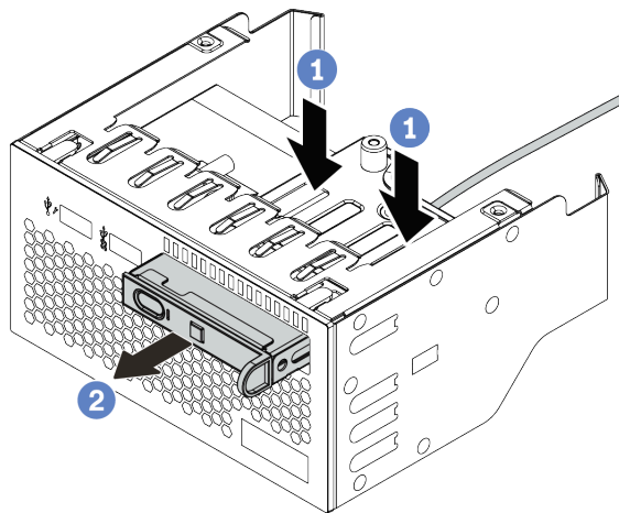
Figura 66. Remoção do painel de diagnóstico LCD
