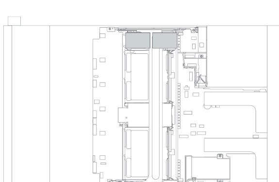
Figura 164. Na gaiola de unidade do meio de 2,5 polegadas
