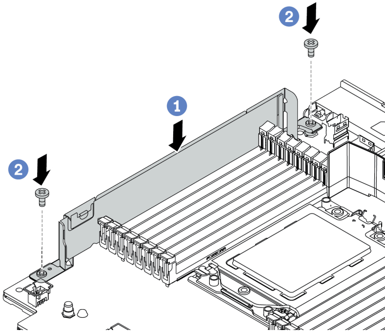
Figura 59. Instalação do retentor de cabo
