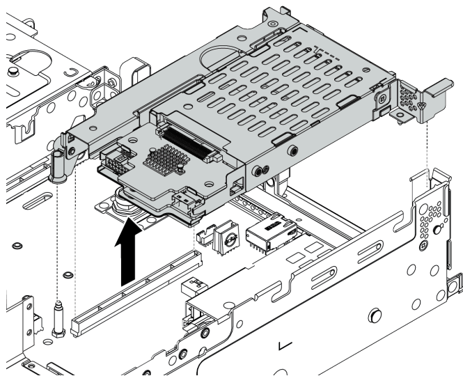
Figura 119. Remoção do conjunto da placa riser
