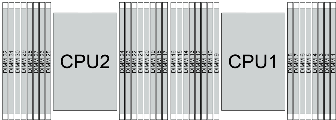
Figura 146. Locais de módulos de memória
