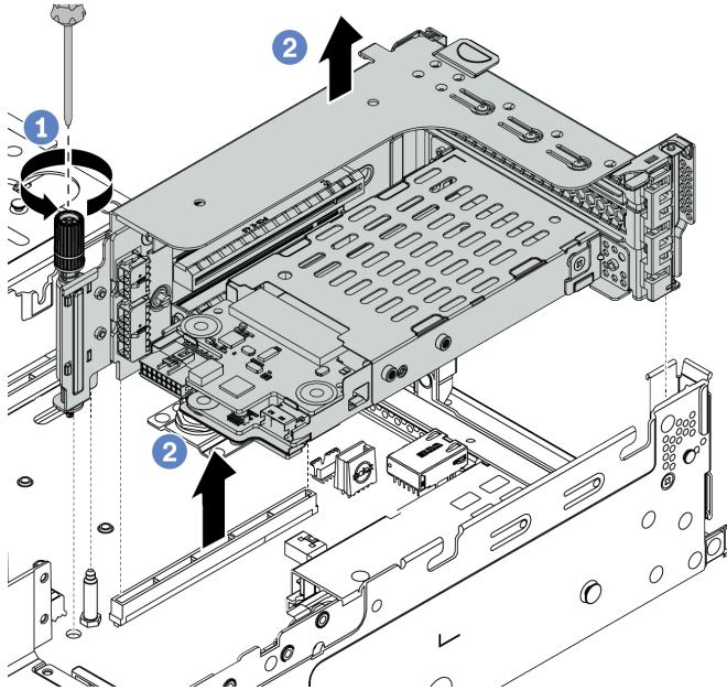
Figura 116. Remoção do conjunto da placa riser
