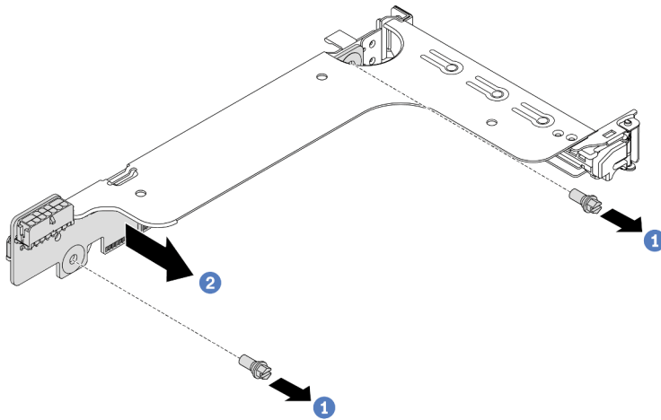
Figura 187. Remoção da placa riser (suporte para placa riser de um ou dois slots)
