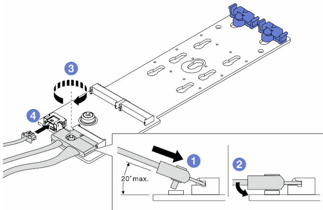
Figura 144. Conectando os cabos M.2
