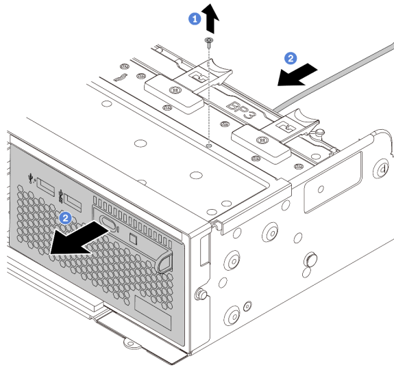
Figura 65. Remoção do conjunto de E/S frontal
