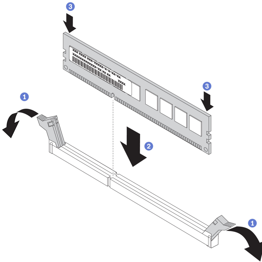
Figura 147. Instalação do módulo de memória
