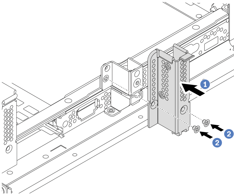
Figura 179. Instalação do suporte de parede traseira B1
