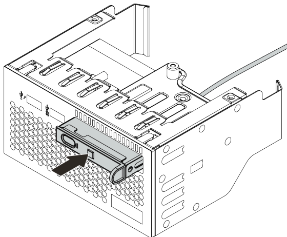
Figura 68. Instalação do painel de diagnóstico LCD
