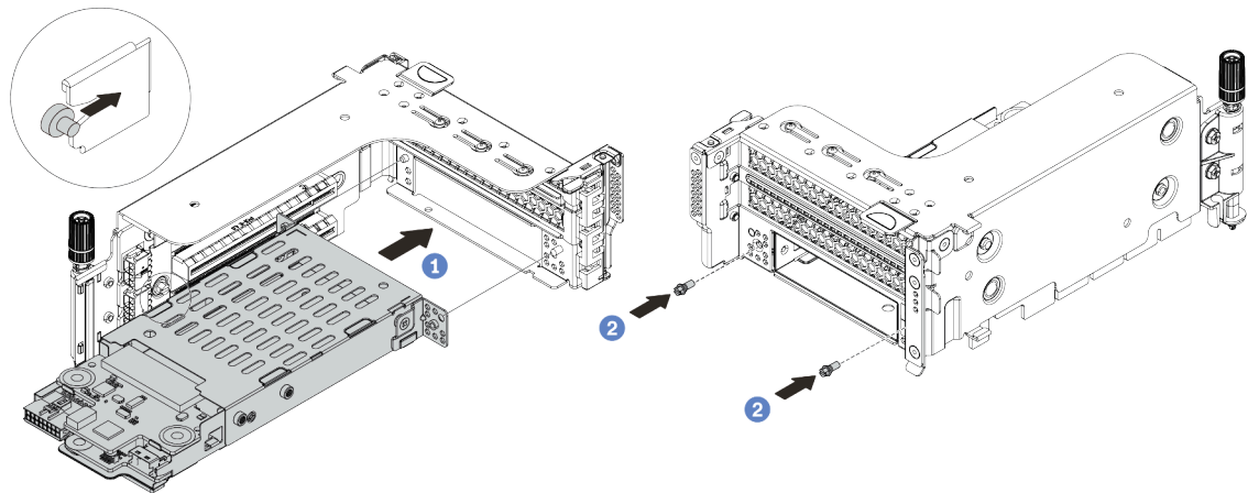
Figura 121. Instalação da gaiola de unidade de 7 mm
