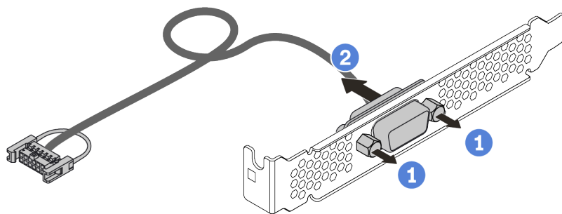
Figura 195. Desmontagem do módulo de porta serial
