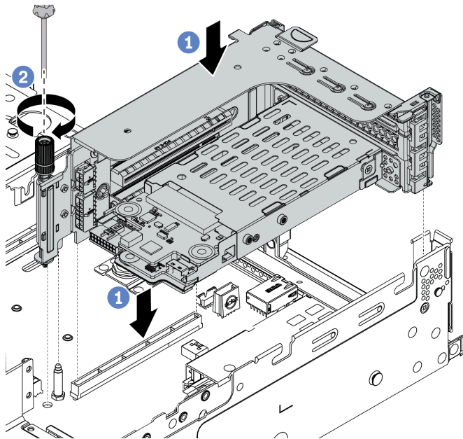
Figura 122. Instalação da gaiola de unidade de 7 mm
