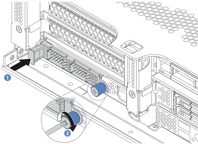
Figura 149. Instalação do adaptador OCP 3.0 Ethernet
