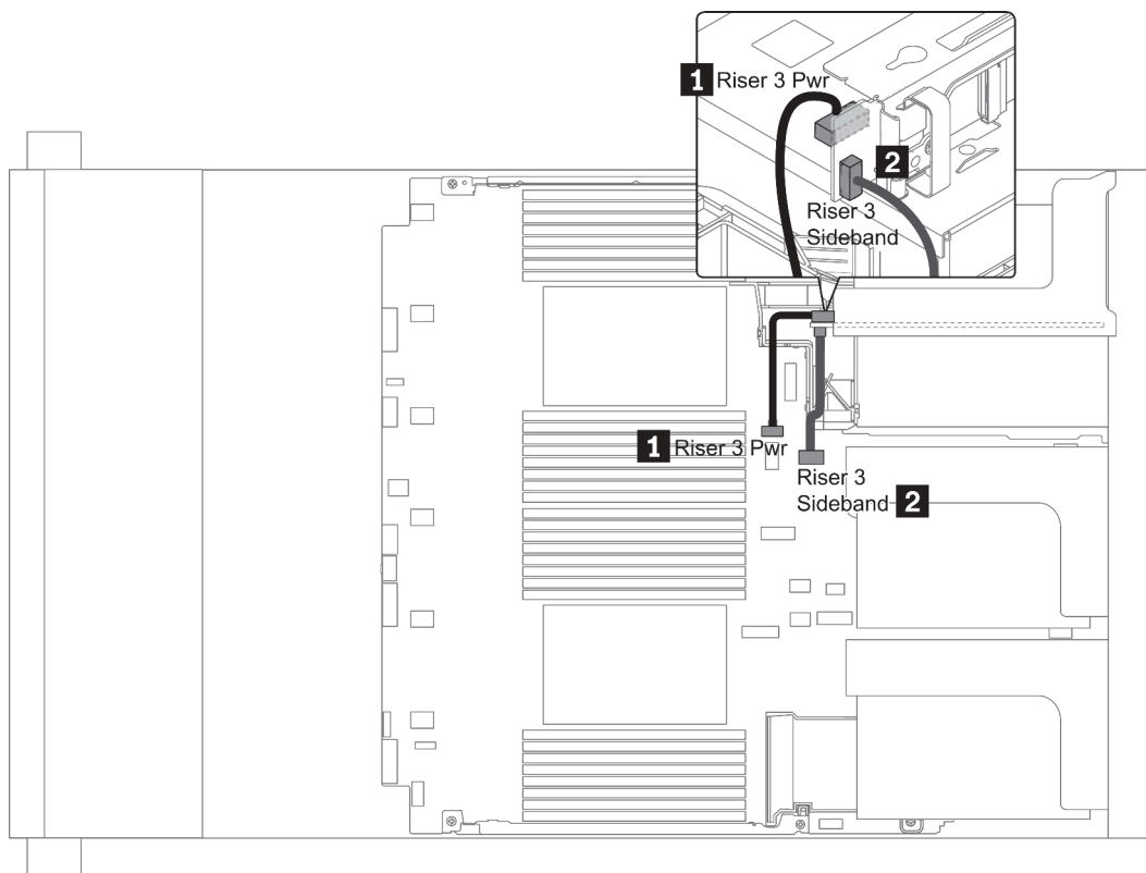
Figura 16. Conexão lateral e de energia da placa riser 3
