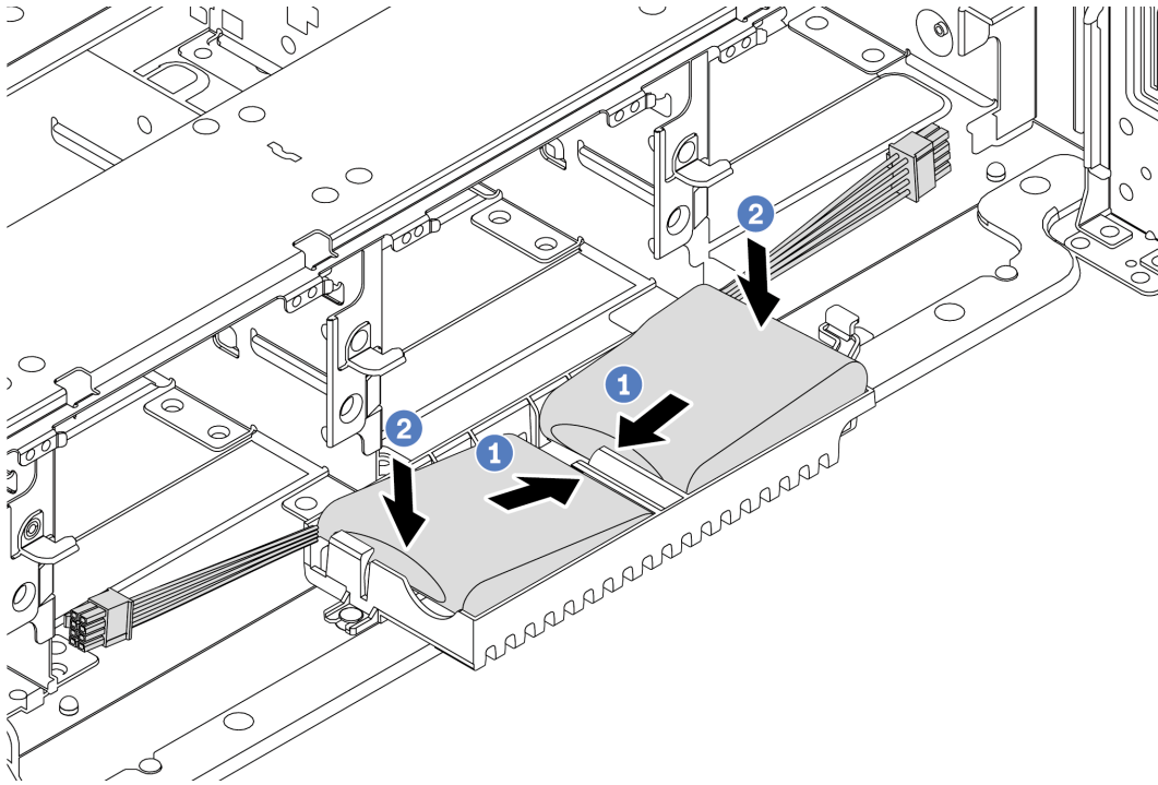
Figura 175. Instalação do módulo de supercapacitor
