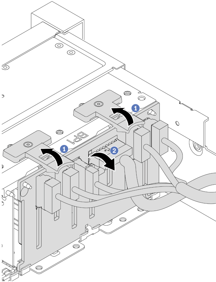
Figura 81. Remoção do painel traseiro da unidade de 2,5 polegadas
