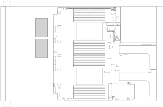
Figura 163. Na placa defletora de ar de GPU
