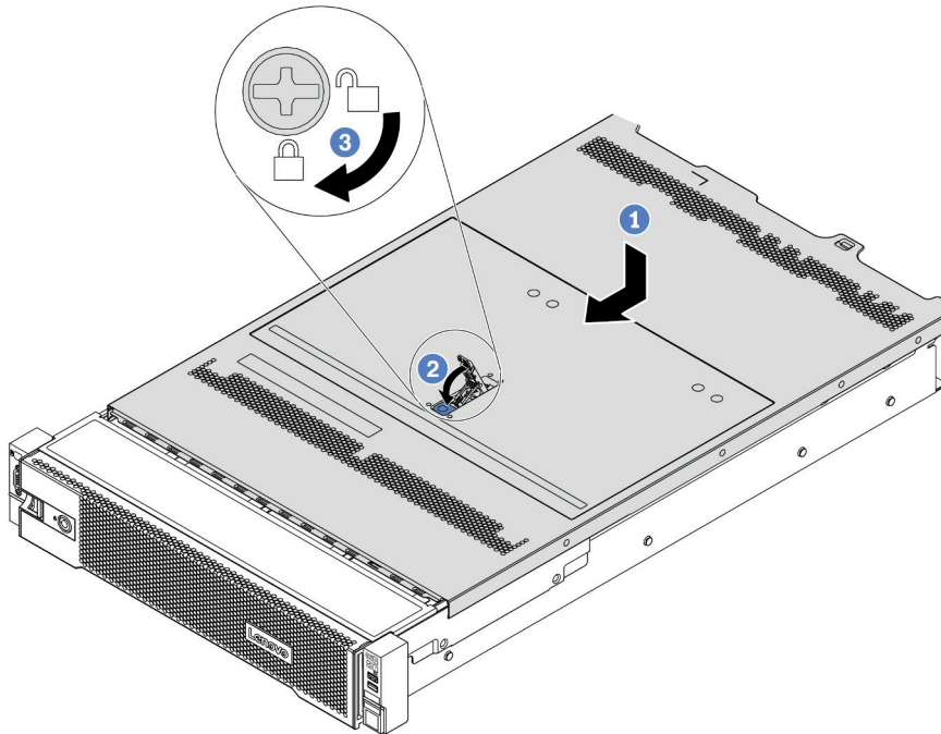
Figura 209. Instalação da tampa superior
