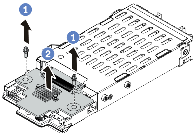
Figura 93. Remoção do painel traseiro da unidade de 7 mm (superior)
