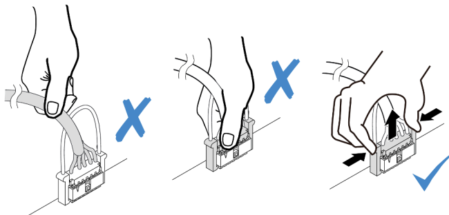
Figura 194. Desconectando o cabo da porta serial
