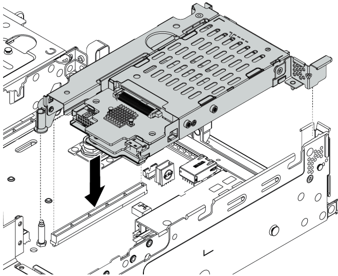
Figura 123. Instalação da gaiola de unidade de 7 mm
