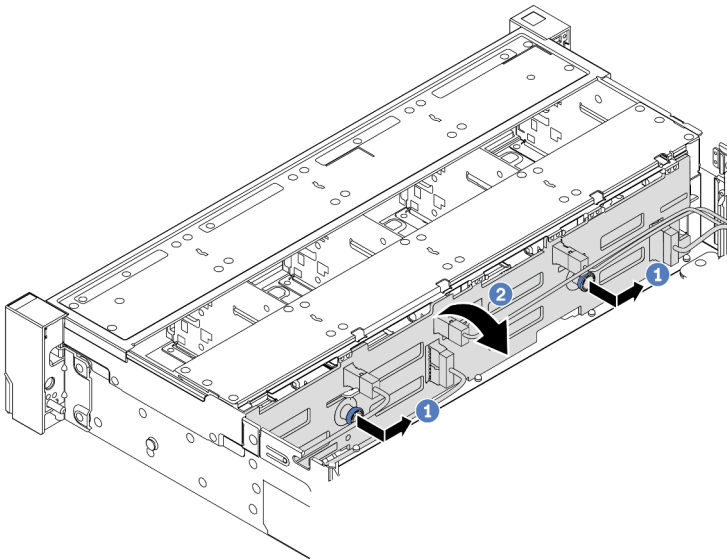
Figura 87. Remoção do painel traseiro da unidade de 3,5 polegadas
