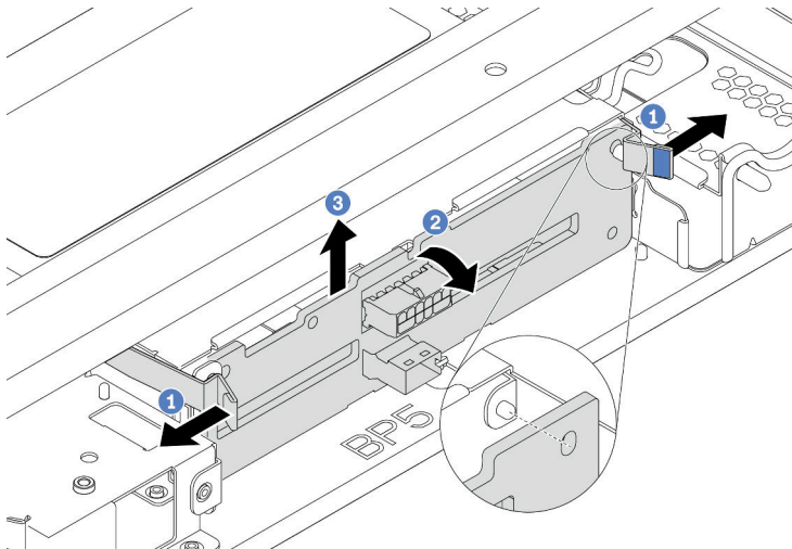
Figura 83. Removendo o painel traseiro da unidade de 4 x 2,5 polegadas
