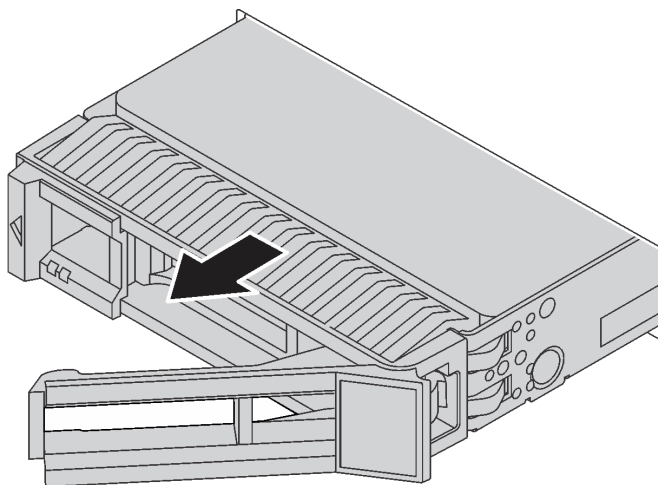
Figura 78. Remoção da unidade hot-swap
