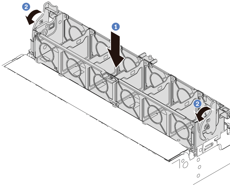
Figura 205. Instalação do compartimento do ventilador do sistema
