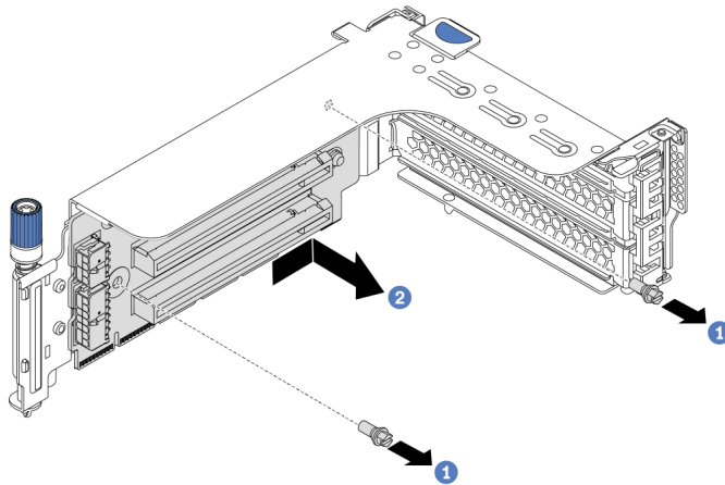
Figura 186. Remoção da placa riser (suporte para placa riser de três slots)
