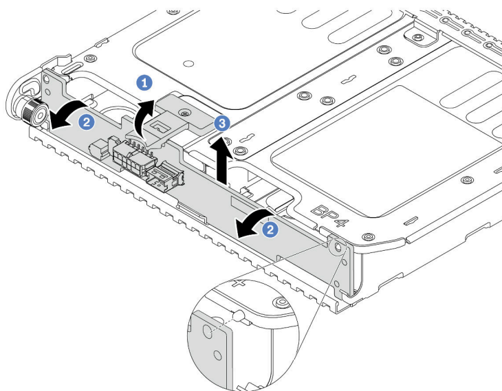
Figura 89. Removendo o painel traseiro da unidade de 2 x 3,5 polegadas
