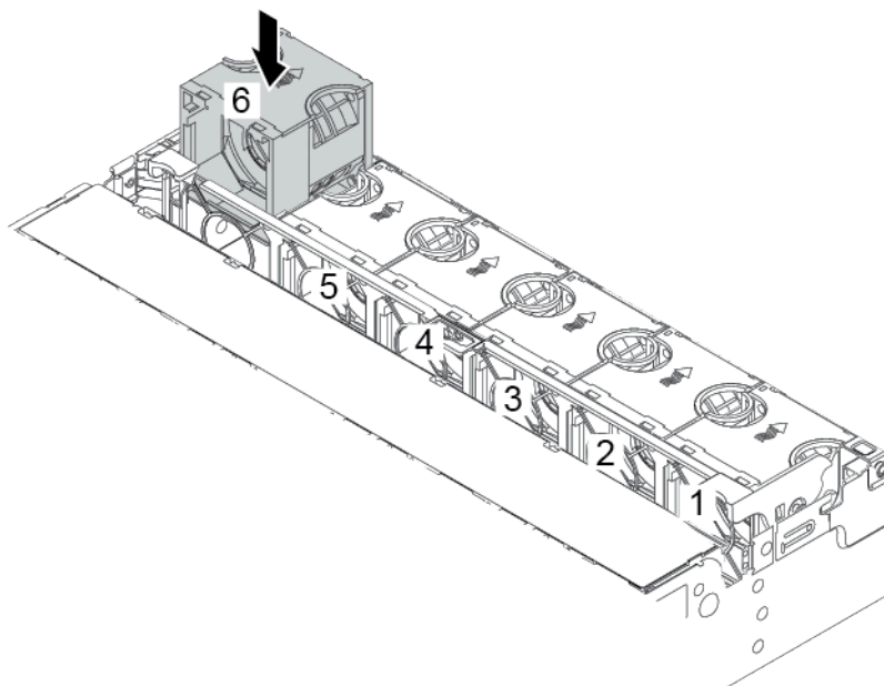
Figura 203. Instalação do ventilador do sistema
