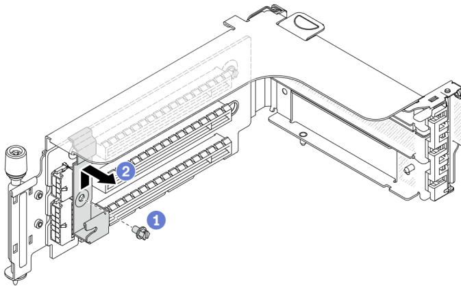
Figura 118. Remoção do clipe de fixação do compartimento da unidade de 7 mm
