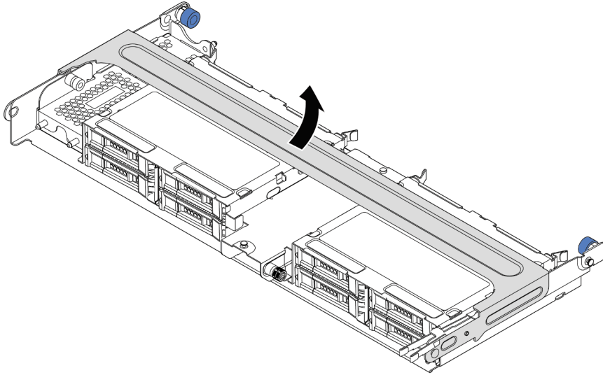
Figura 167. Abrindo a alça da gaiola de unidade do meio
