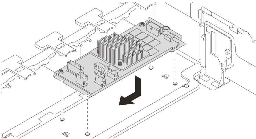
Figura 130. Instalação do adaptador HBA/RAID de CFF interno
