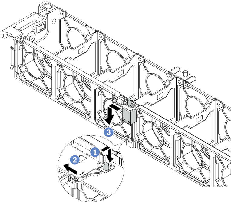
Figura 131. Remoção da chave de intrusão
