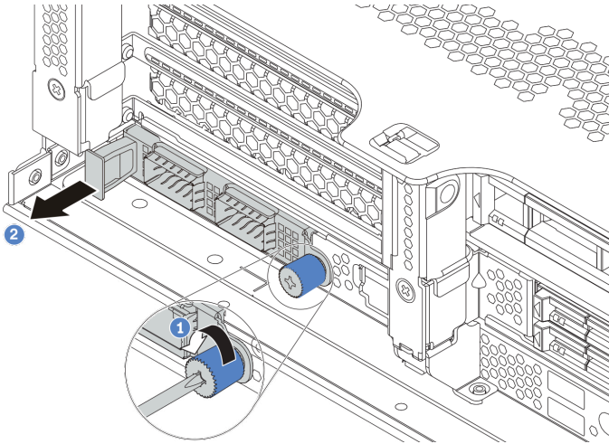
Figura 148. Remoção do adaptador OCP 3.0 Ethernet
