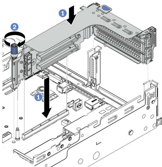
Figura 191. Instalação do conjunto de 1/2 placa riser (suporte para placa riser de três slots)
