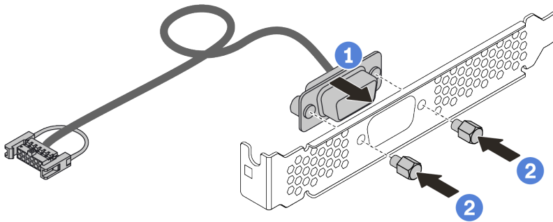
Figura 196. Montagem do módulo de porta serial
