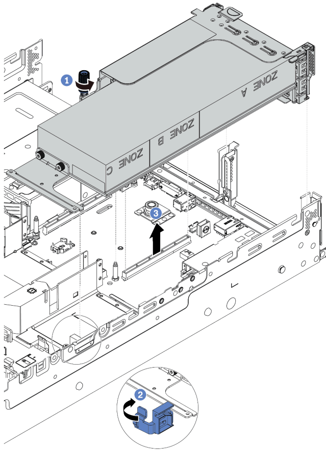
Figura 69. Removendo o conjunto de placa riser
