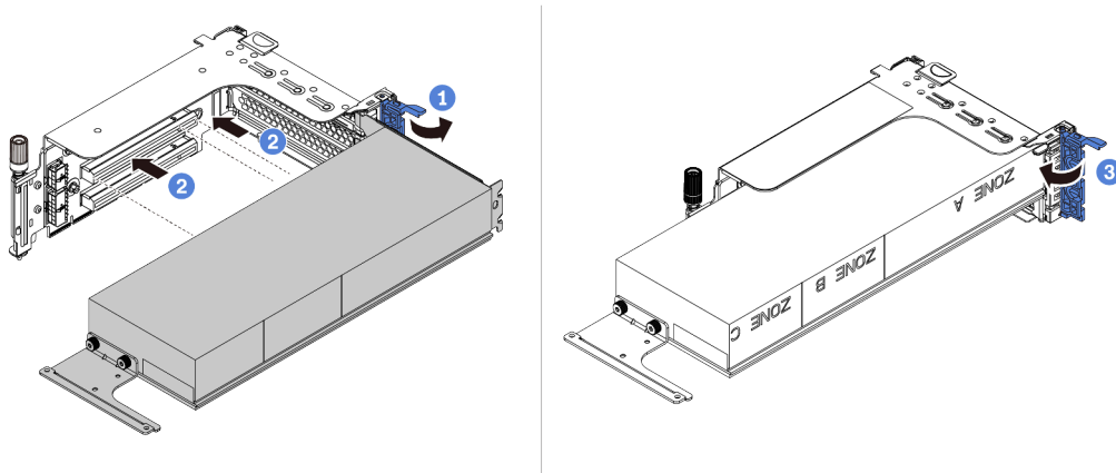
Figura 74. Instalando o adaptador de GPU no compartimento da placa riser
