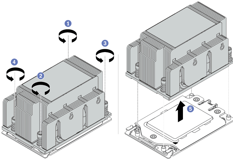
Figura 210. Removendo um dissipador de calor padrão
