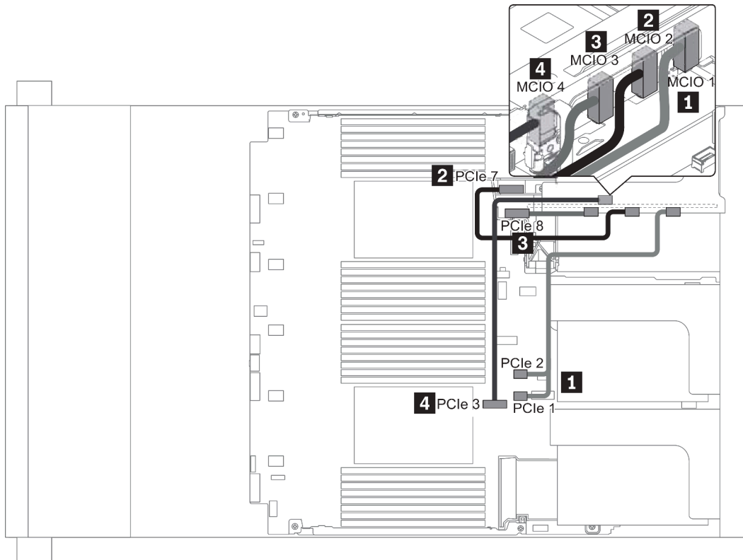
Figura 17. Roteamento de cabos da placa riser 3 (PCIe x8/x8 ou x16/x16)
