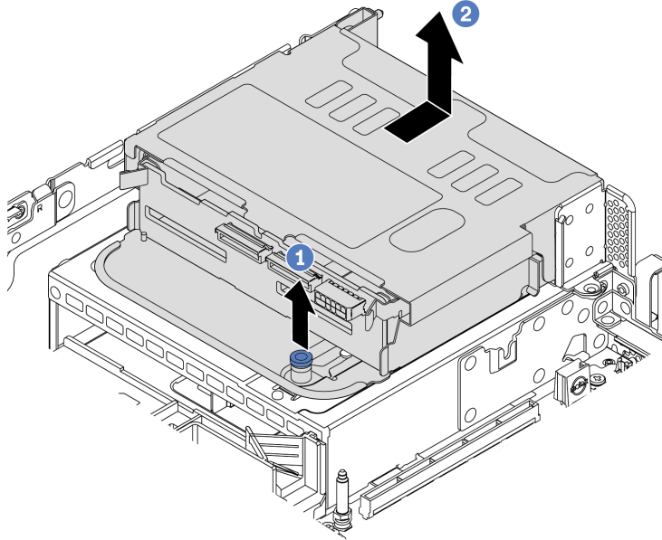
Figura 112. Removendo a gaiola de unidade traseira de 4 x 2,5 polegadas
