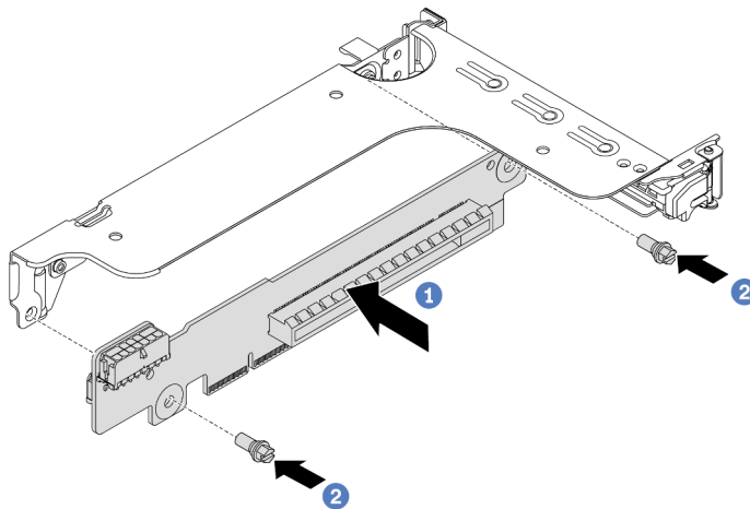
Figura 189. Instalação da placa riser (suporte para placa riser de um ou dois slots)
