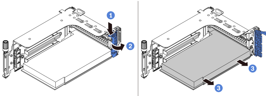
Figura 185. Remoção do adaptador PCIe
