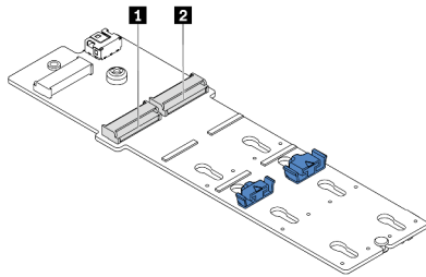
Figura 141. Slot da unidade M.2
