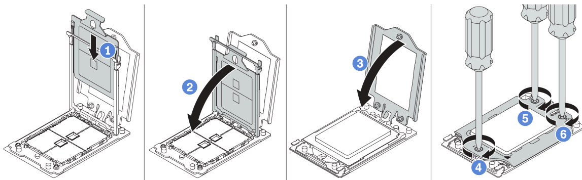
Figura 213. Instalação do processador
