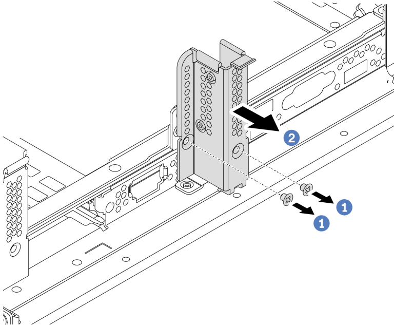
Figura 178. Remoção do suporte de parede traseira B1
