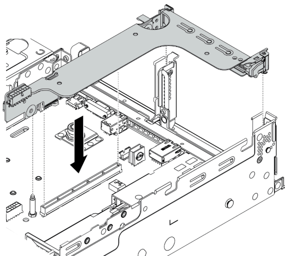
Figura 192. Instalação do conjunto de 1/2 placa riser (suporte para placa riser de um slot)
