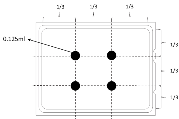
Figura 214. Aplicando graxa térmica
