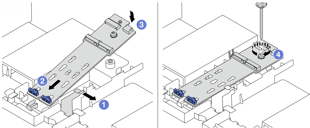
Figura 142. Instalação do adaptador M.2
