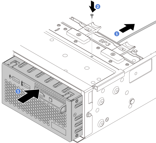
Figura 67. Instalação do conjunto de E/S frontal
