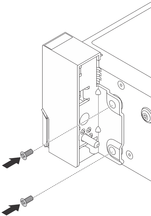
Figura 158. Instalação de parafusos
