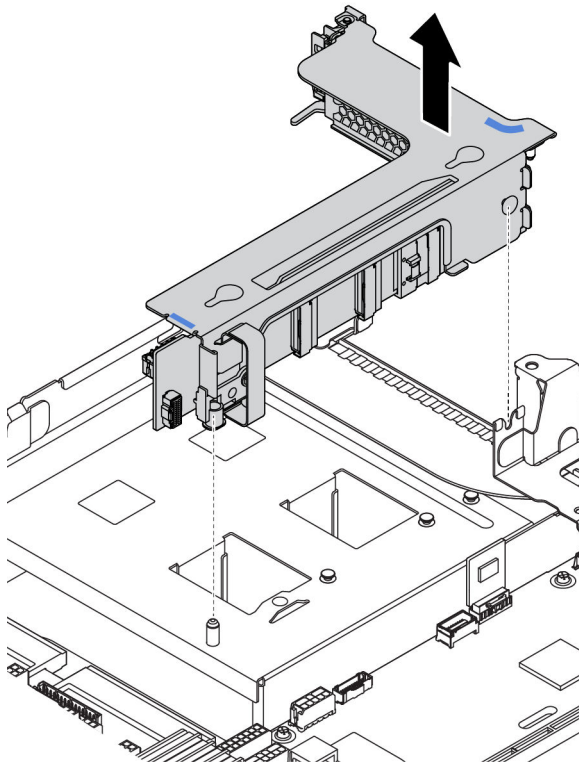
Figura 184. Remoção do conjunto de placa riser 3 (suporte para placa riser de dois slots)
