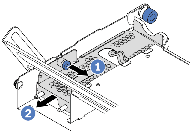
Figura 170. Removendo a tampa de metal
