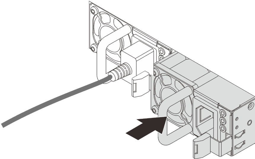
Figura 128. Instalação da fonte de alimentação hot-swap
