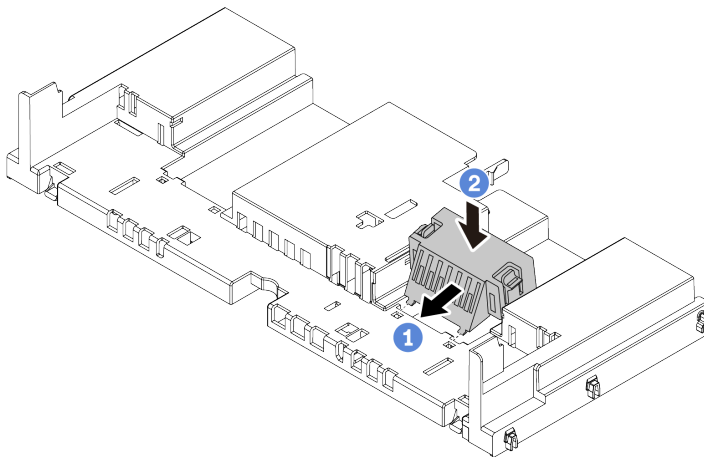
Figura 56. Instalando os preenchimentos no defletor de ar padrão
