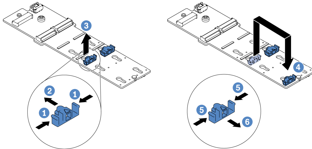
Figura 140. Ajuste do retentor M.2
