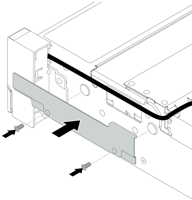
Figura 159. Instalação do retentor de cabos
