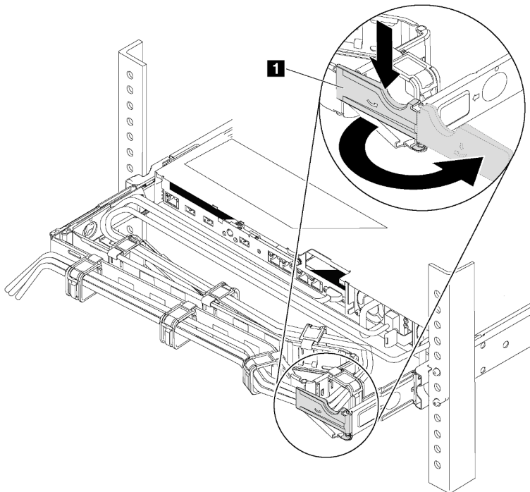
Figura 124. Ajuste do CMA
