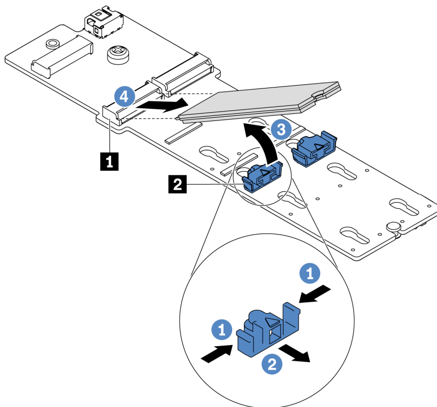
Figura 138. Remoção da unidade M.2
