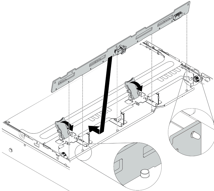
Figura 92. Instalação do painel traseiro da unidade de 4 x 3,5 polegadas
