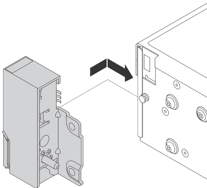
Figura 157. Instalação da trava do rack
