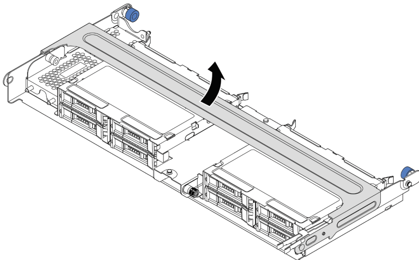
Figura 169. Abrindo a alça da gaiola de unidade do meio
