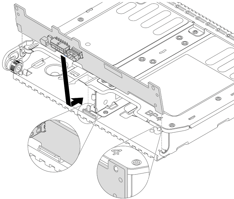
Figura 91. Instalação do painel traseiro da unidade de 2 x 3,5 polegadas
