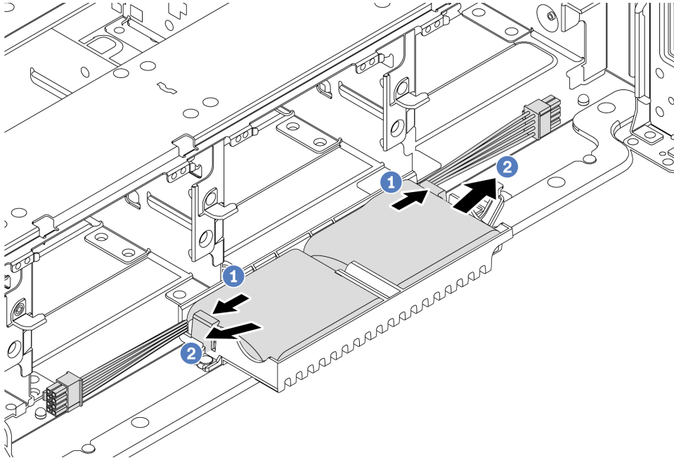
Figura 172. Remoção do módulo de supercapacitor
