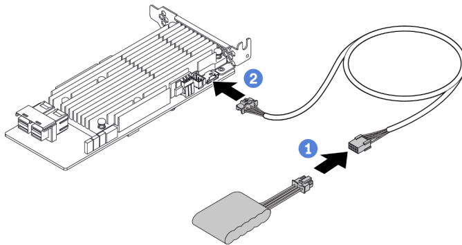
Figura 18. Conectando o módulo de supercapacitor RAID ao adaptador RAID
