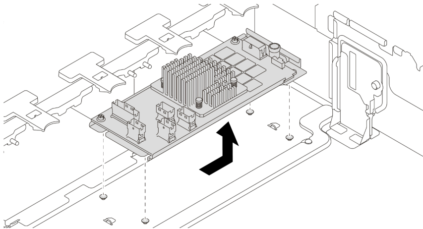
Figura 129. Remoção do adaptador de expansor CFF RAID/HBA/RAID interno
