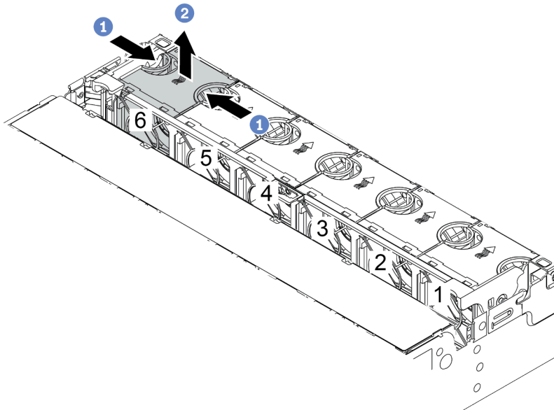
Figura 202. Remoção do ventilador do sistema
