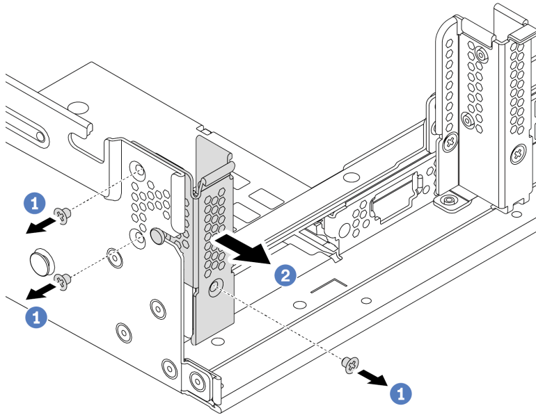
Figura 176. Instalação do suporte de parede traseira A1
