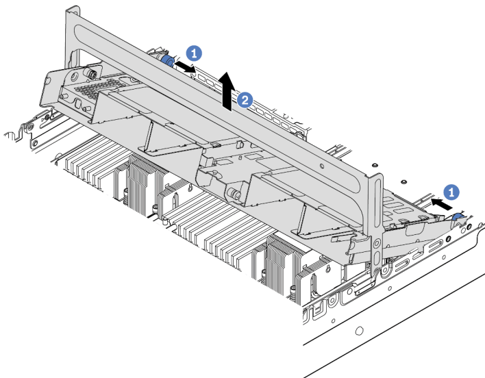
Figura 98. Removendo a gaiola de unidade do meio de 2,5 polegadas
