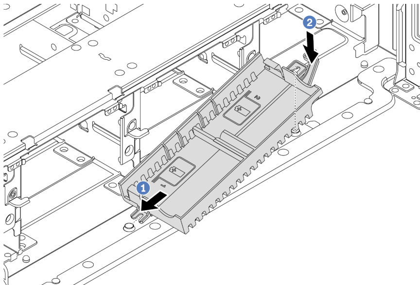
Figura 174. Instalação da caixa do supercapacitor
