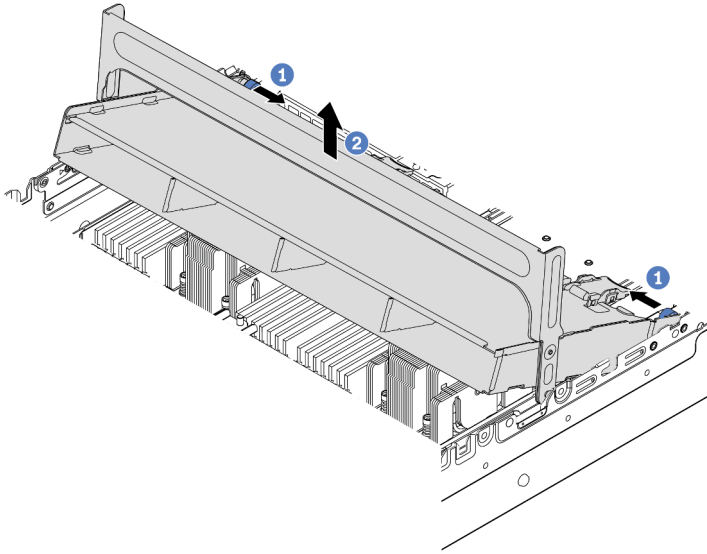
Figura 103. Removendo a gaiola de unidade do meio de 3,5 polegadas
