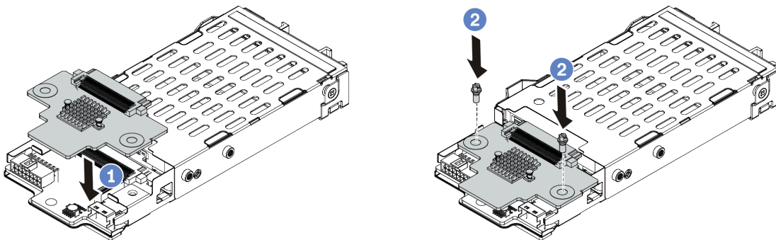
Figura 96. Instalação do painel traseiro da unidade de 7 mm (superior)
