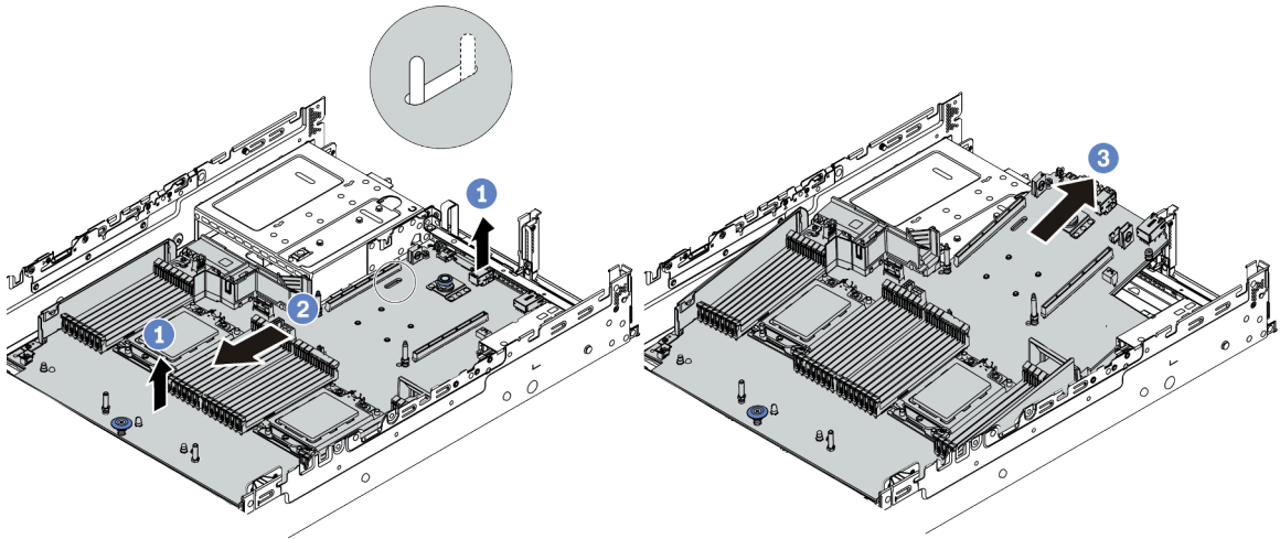
Figura 217. Remoção da placa-mãe
