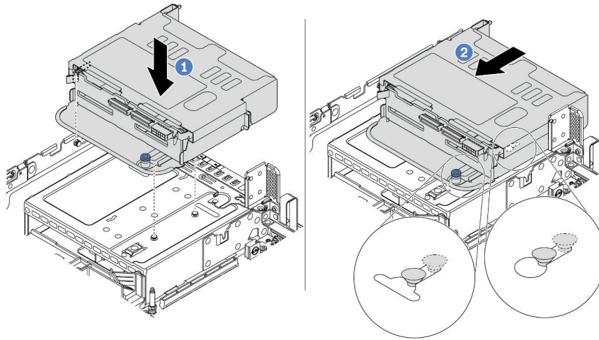
Figura 113. Instalando a gaiola de unidade traseira de 4 x 2,5 polegadas
