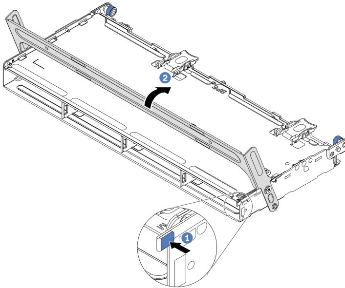
Figura 104. Fechando a alça da gaiola de unidade do meio de 3,5 polegadas
