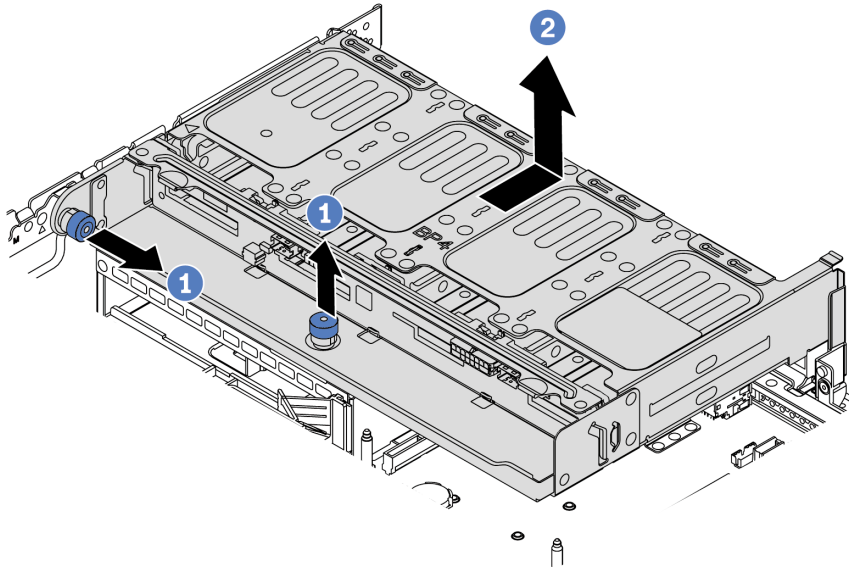
Figura 114. Removendo a gaiola de unidade traseira de 8 x 2,5 polegadas
