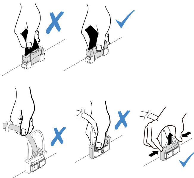
Figura 64. Desconectando os cabos do conjunto de E/S frontal
