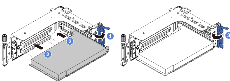
Figura 190. Instalação do adaptador PCIe
