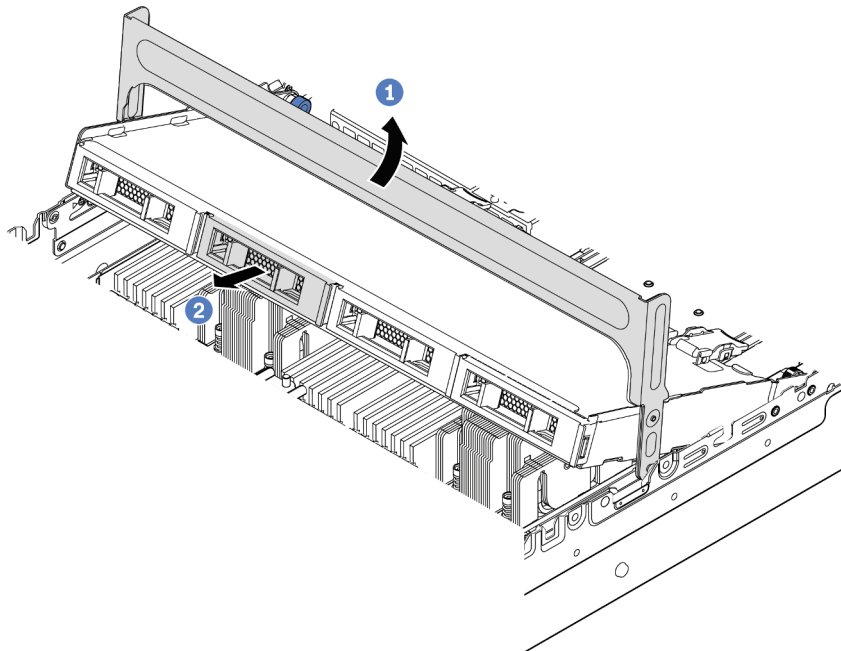
Figura 102. Abrindo a alça da gaiola de unidade e removendo as unidades
