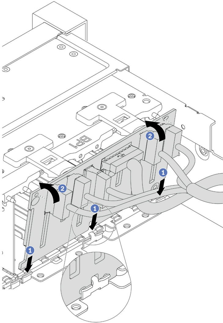
Figura 82. Instalação do backplane da unidade de 2,5 polegadas
