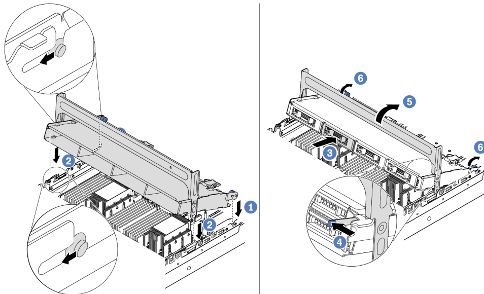
Figura 106. Instalando a gaiola de unidade do meio de 3,5 polegadas e as unidades
