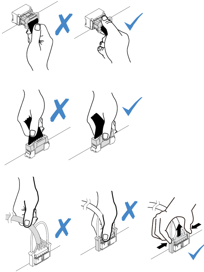
Figura 153. Desconectando os cabos VGA e do conjunto de E/S frontal
