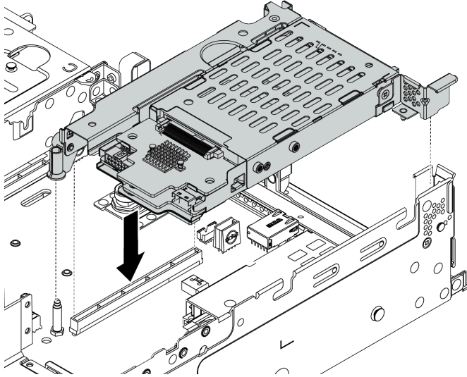
图 123. 安装 7 毫米硬盘仓
