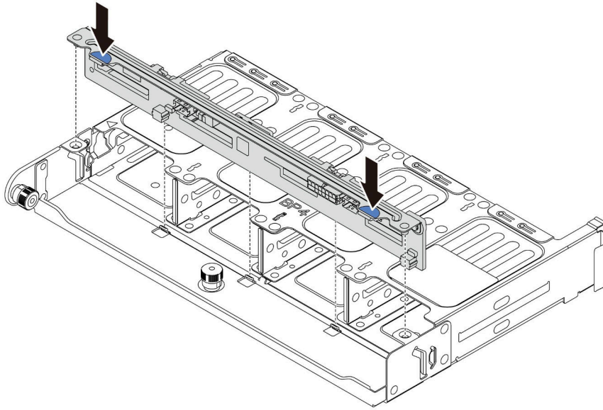
图 86. 安装 8 x 2.5 英寸硬盘背板
