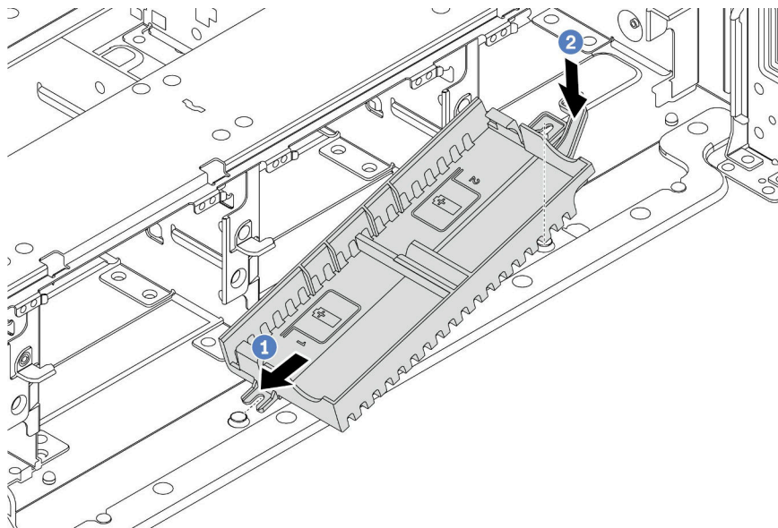
图 174. 安装超级电容器盒
