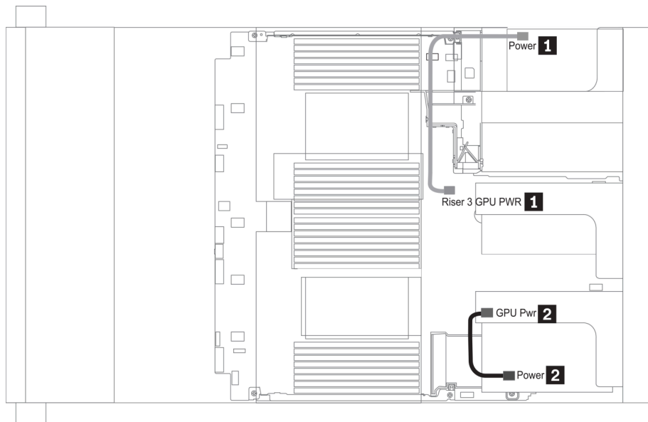
图 15. GPU cable routing
