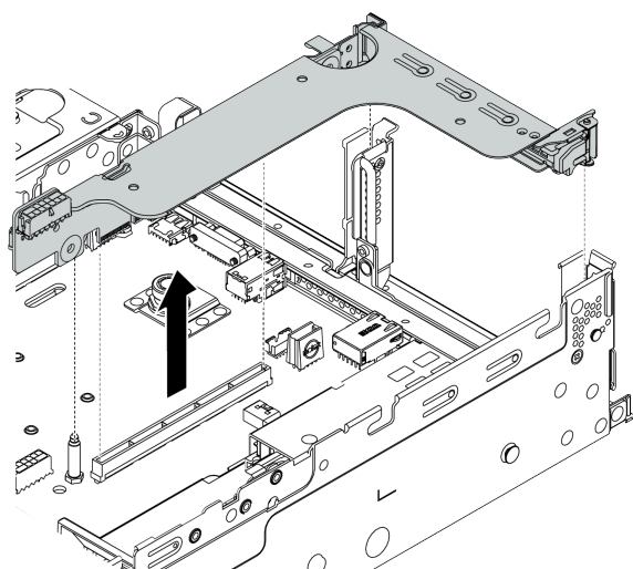
图 183. 卸下转接卡 1/2 组合件 (单插槽转接卡支架)
