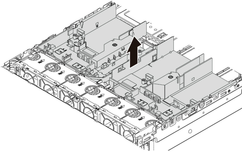
图 54. 卸下 GPU 导风罩
