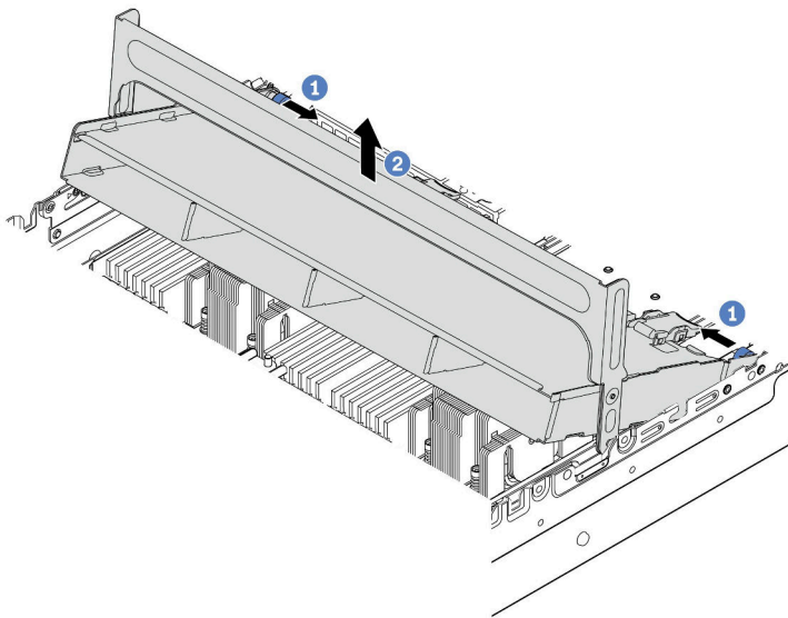
图 103. 卸下中间 3.5 英寸硬盘仓
