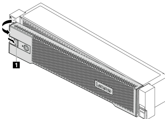
图 198. 卸下安全挡板
