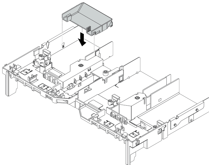
图 73. 安装 GPU 附加导风罩
