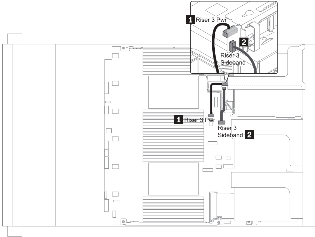
图 16. 转接卡 3 电源和边带连接
