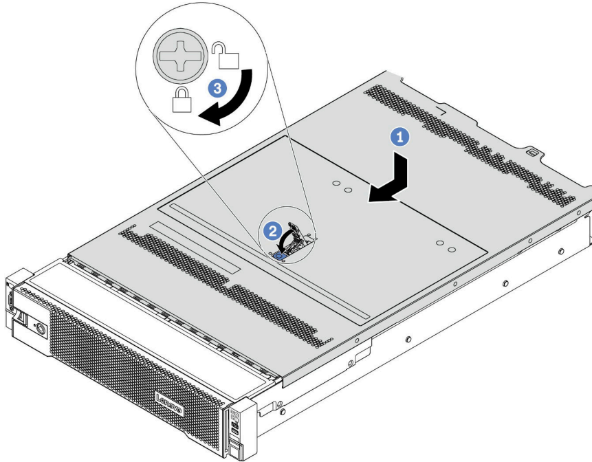
图 209. 安装顶盖
