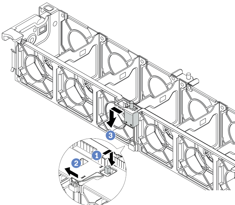
图 131. 卸下入侵感应开关
