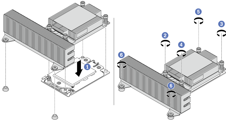
图 216. 安装高性能散热器
