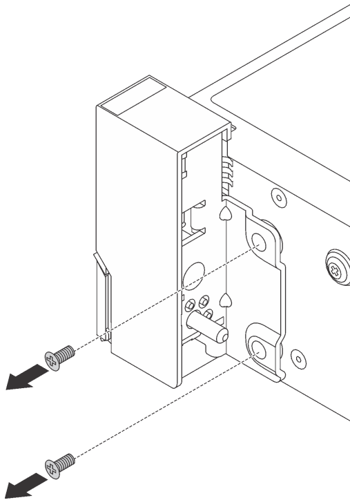
图 155. 卸下螺钉
