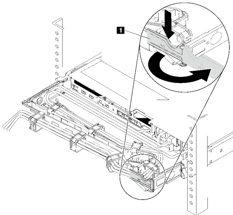
图 124. 调整 CMA
