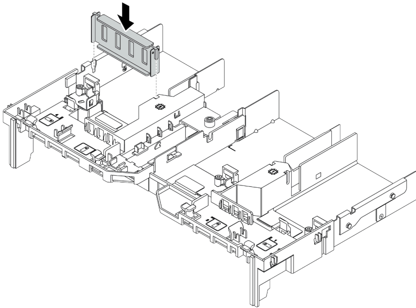
图 76. 安装 GPU 填充件
