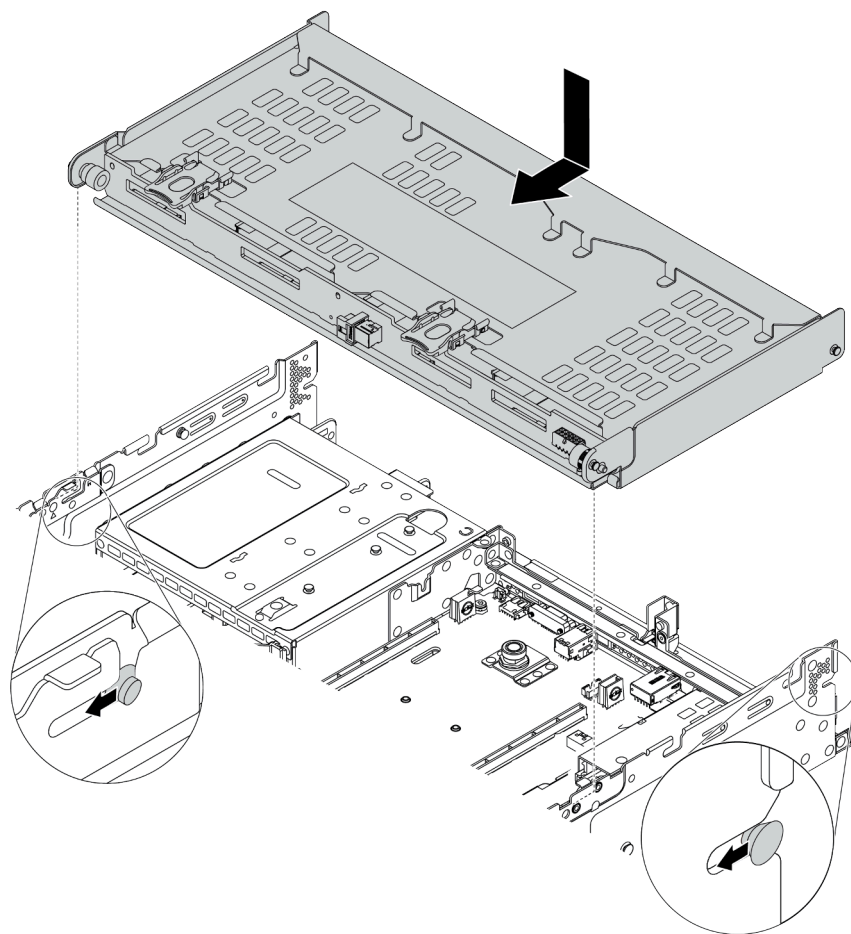
图 110. 安装 4 x 3.5 英寸背面硬盘仓
