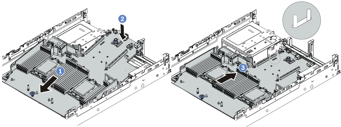
图 218. 安装主板
