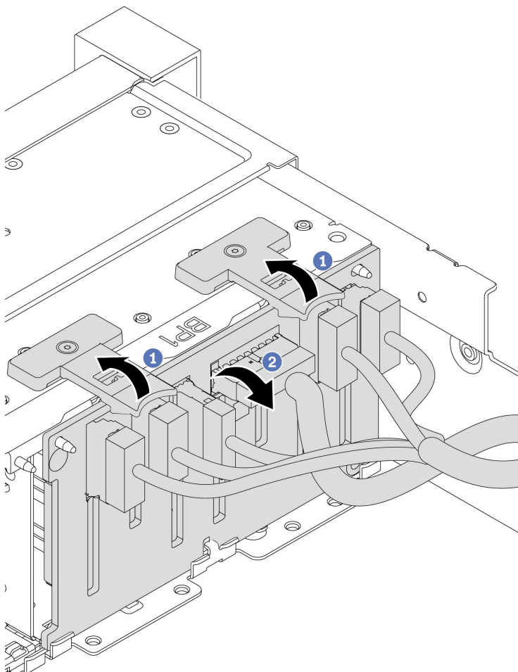
图 81. 卸下 2.5 英寸硬盘背板
