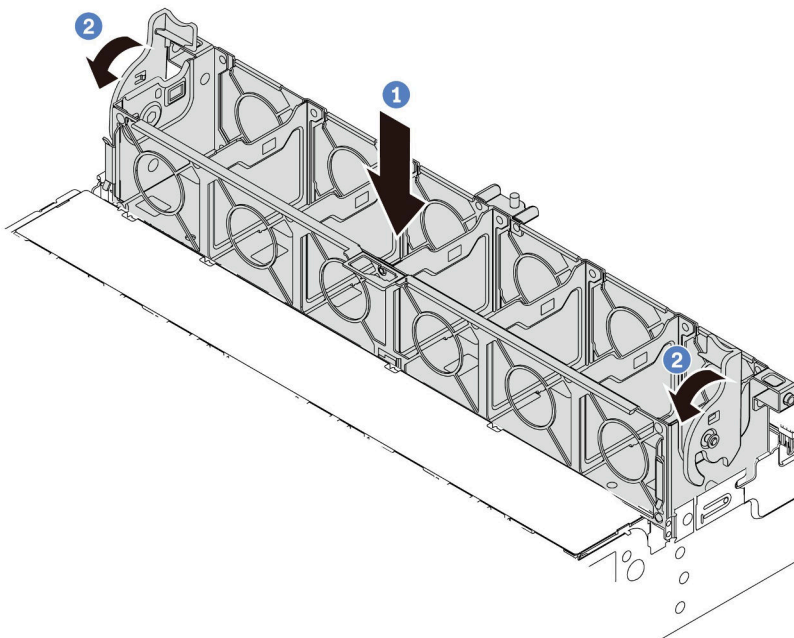
图 205. 安装系统风扇架
