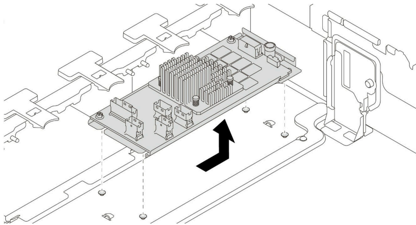
图 129. 卸下内部 CFF RAID/HBA/RAID 扩展器适配器
