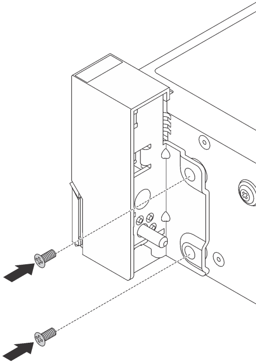
图 158. 螺钉安装
