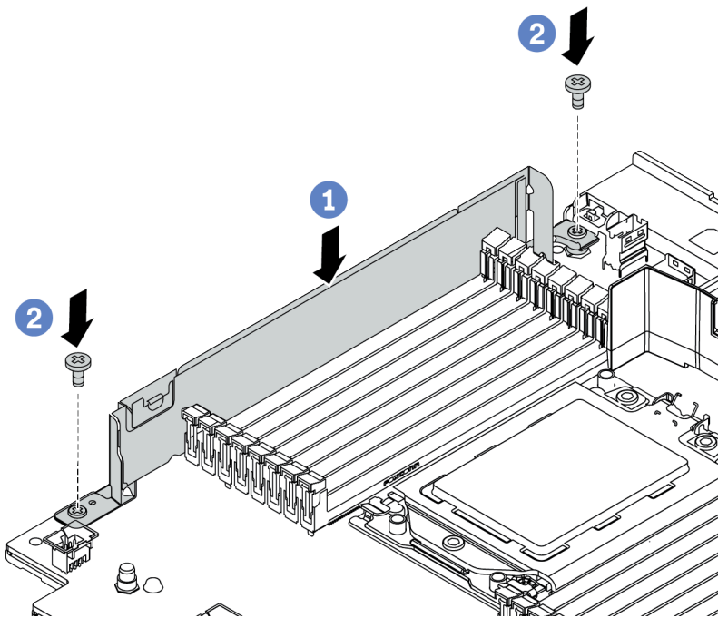
图 59. 安装线缆固定扣
