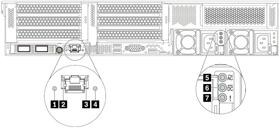
图 10. 服务器的后视图 LED
