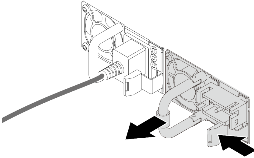
图 125. 卸下热插拔电源模块
