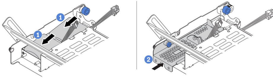
图 171. 安装超级电容器模块
