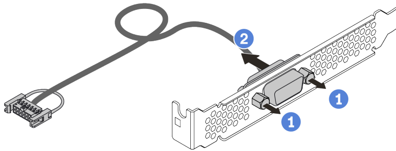
图 195. 拆卸串口模块
