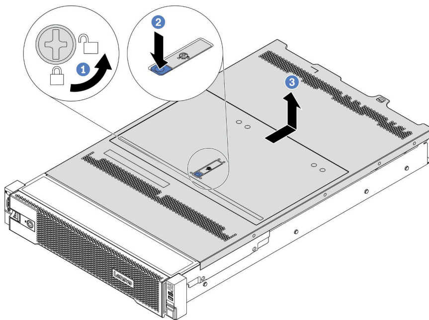
图 206. 卸下顶盖
