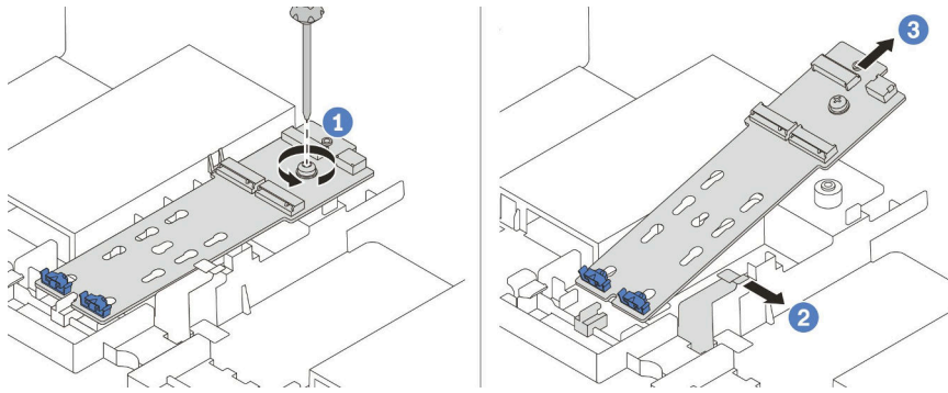
图 139. 卸下 M.2 适配器
