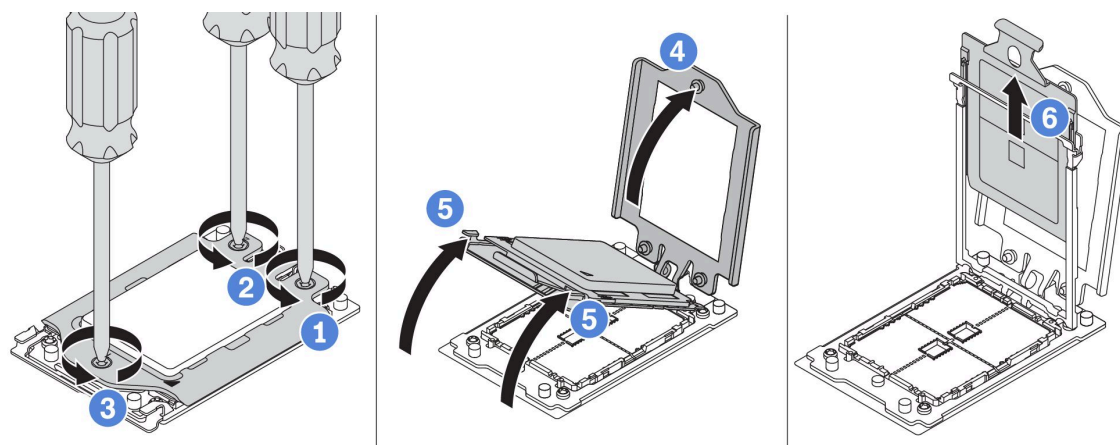
图 212. 卸下处理器
