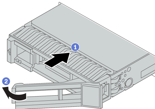
图 80. 安装热插拔硬盘
