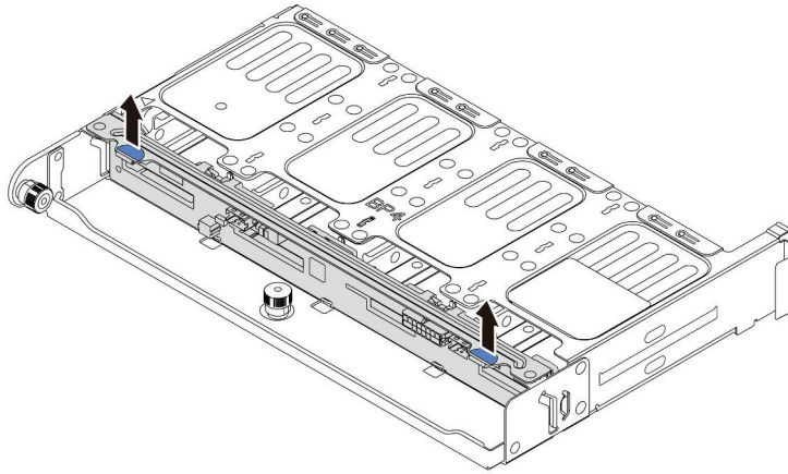
图 84. 卸下 8 x 2.5 英寸硬盘背板
