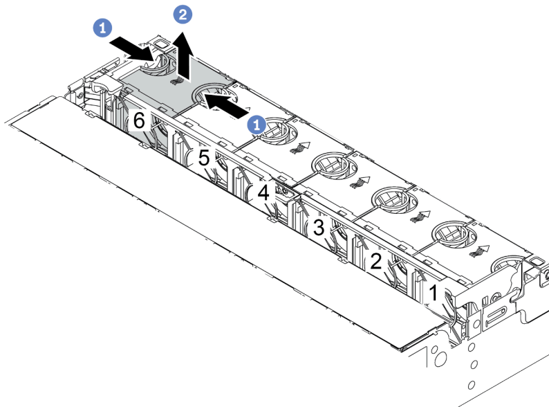
图 202. 卸下系统风扇
