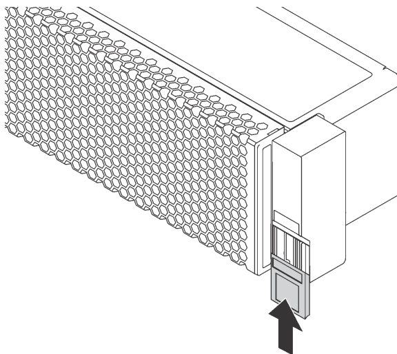
图 160. 安装标识标签板
