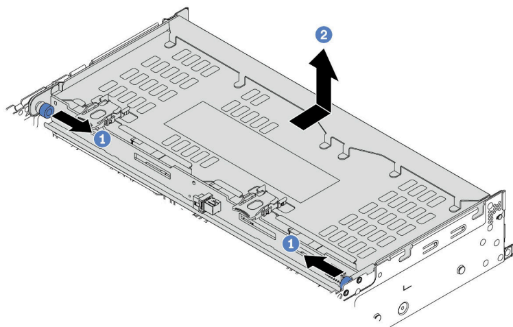
图 109. 卸下 4 x 3.5 英寸背面硬盘仓
