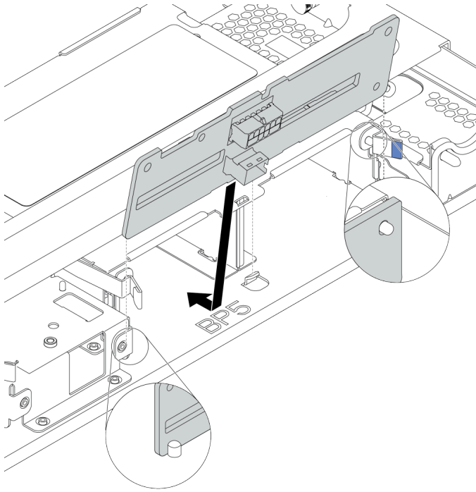
图 100. 安装背板
