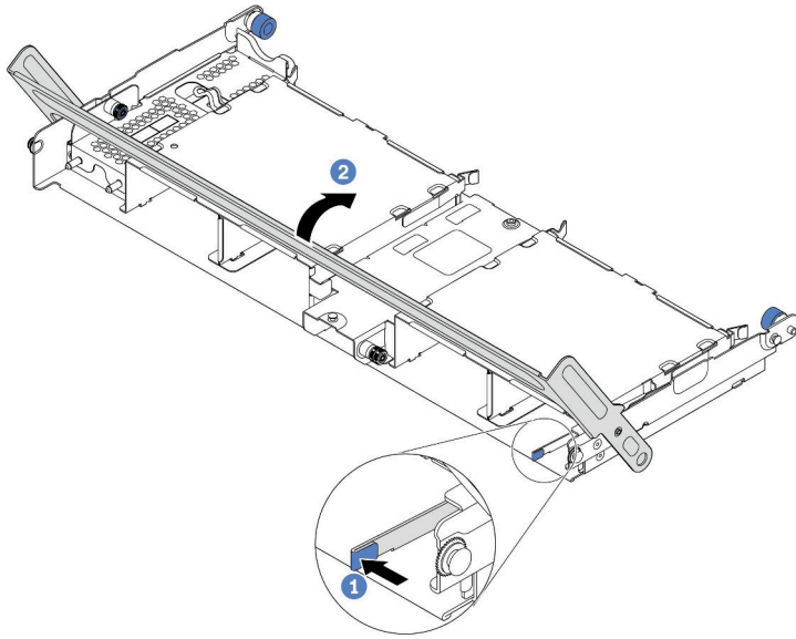
图 99. 合上中间 2.5 英寸硬盘仓的手柄
