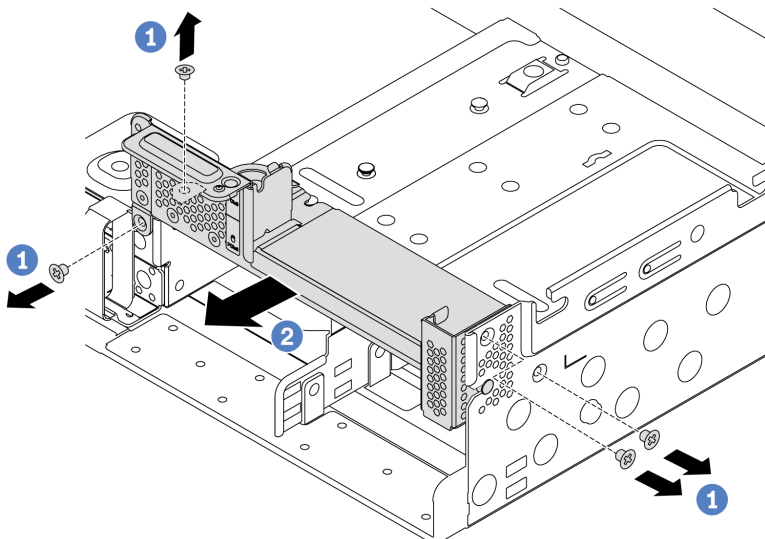
图 180. 卸下 C1 后壁支架
