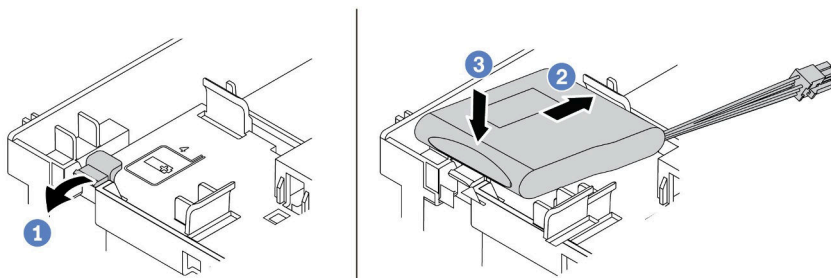
图 166. 导风罩上的超级电容器安装
