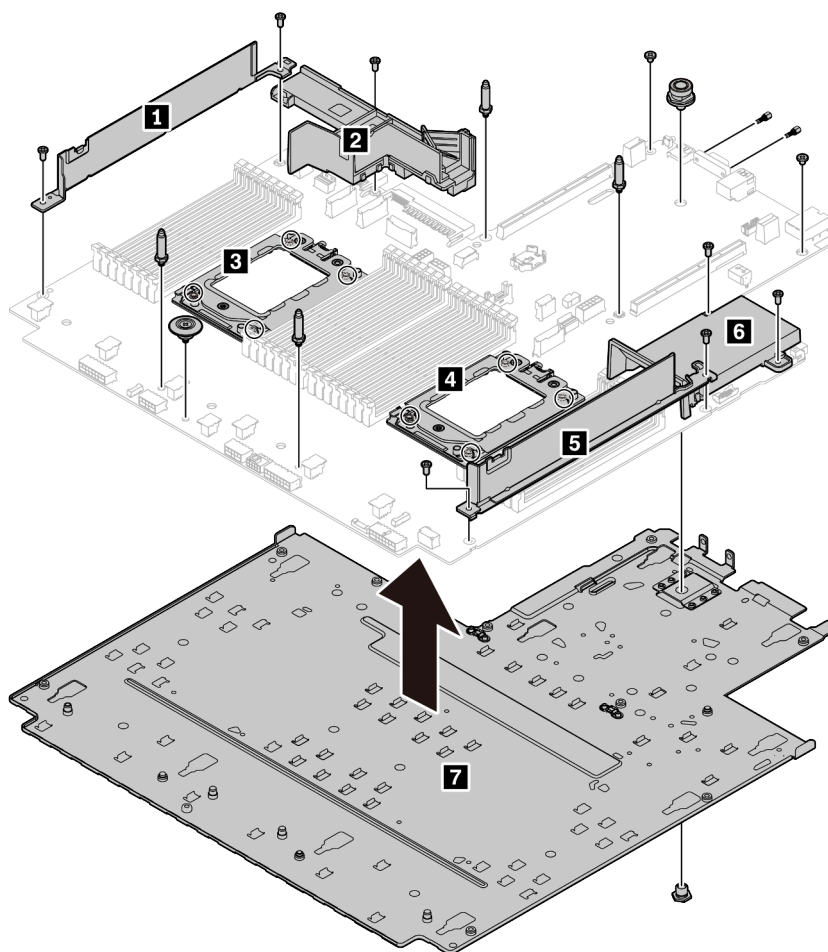
图 220. 拆卸主板
