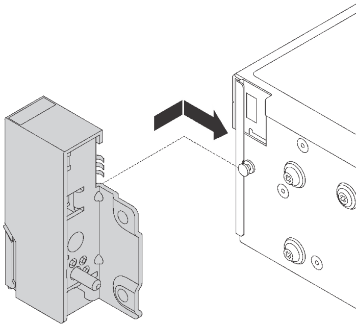
图 157. 安装机架滑锁
