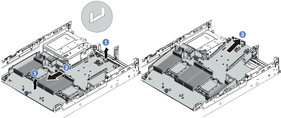
图 217. 卸下主板
