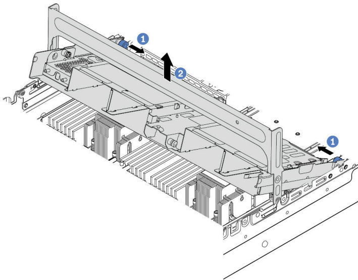
图 98. 卸下中间 2.5 英寸硬盘仓
