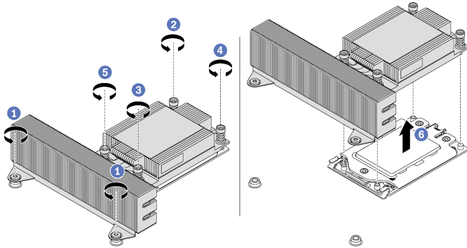
图 211. 卸下高性能散热器
