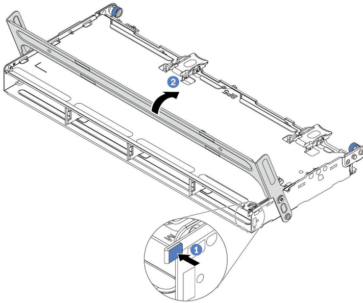
图 104. 合上中间 3.5 英寸硬盘仓的手柄
