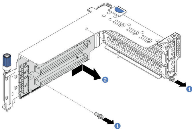
图 186. 卸下转接卡（三插槽转接卡支架）
