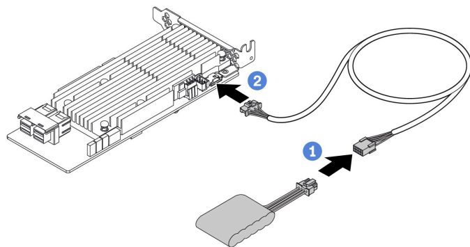
图 18. 将 RAID 超级电容器模块连接到 RAID 适配器
