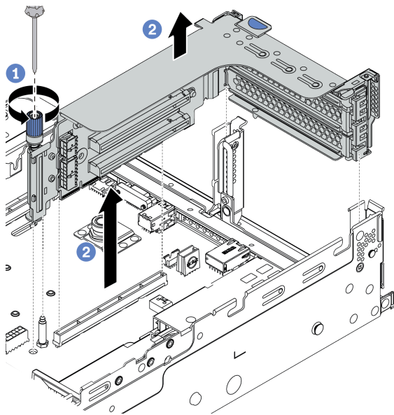
图 182. 卸下转接卡 1/2 组合件（三插槽支架）
