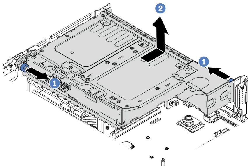
图 107. 卸下 2 x 3.5 英寸背面硬盘仓
