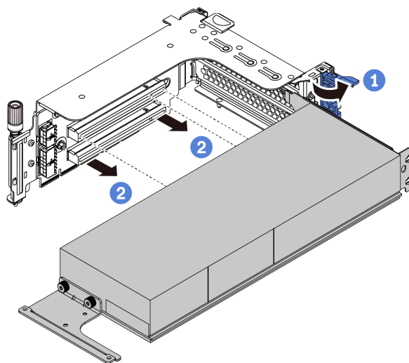
图 70. 卸下 GPU 适配器
