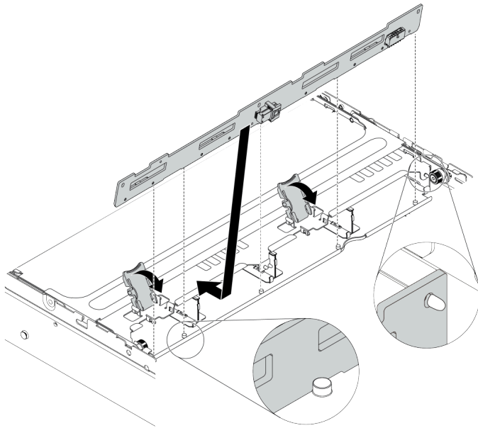
图 105. 安装背板
