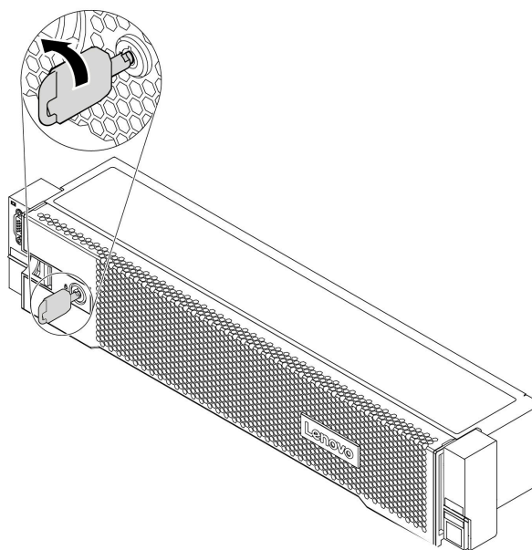
图 201. 锁定安全挡板
