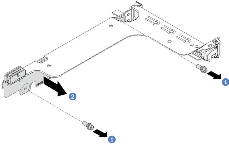
图 187. 卸下转接卡（单插槽或双插槽转接卡支架）
