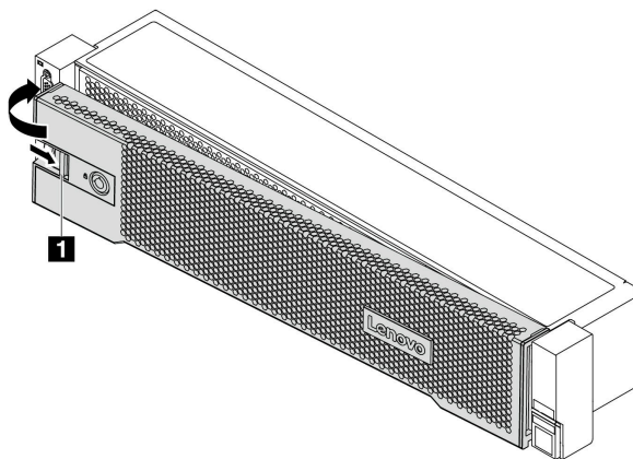
图 200. 安装安全挡板
