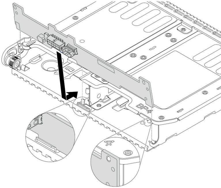
图 91. 安装 2 x 3.5 英寸硬盘背板
