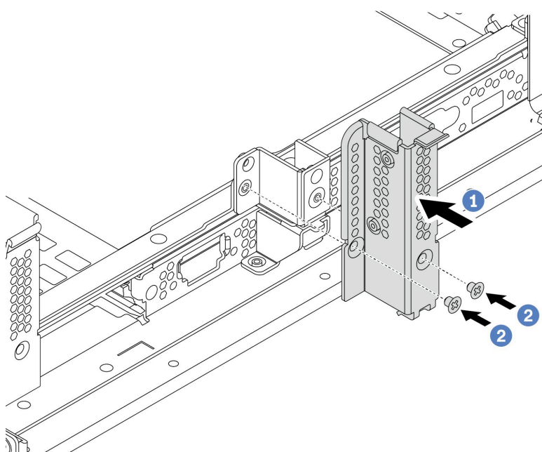
图 179. B1 背面壁挂支架安装
