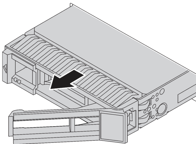
图 78. 卸下热插拔硬盘
