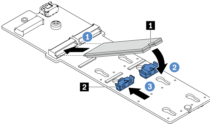
图 143. 安装 M.2 硬盘
