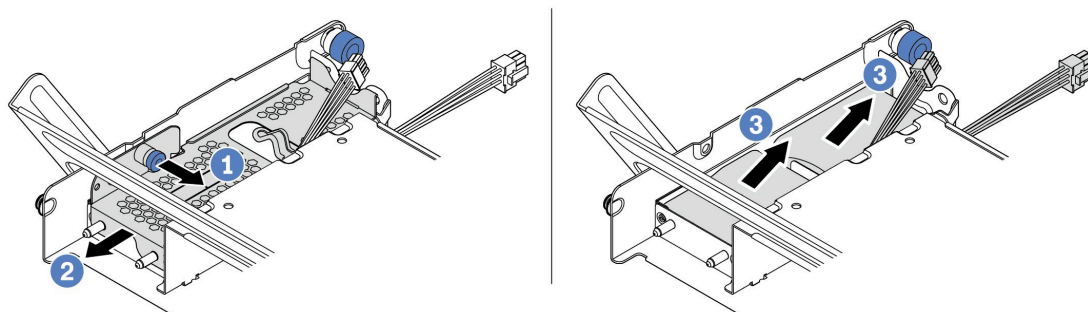
图 168. 卸下超级电容器模块
