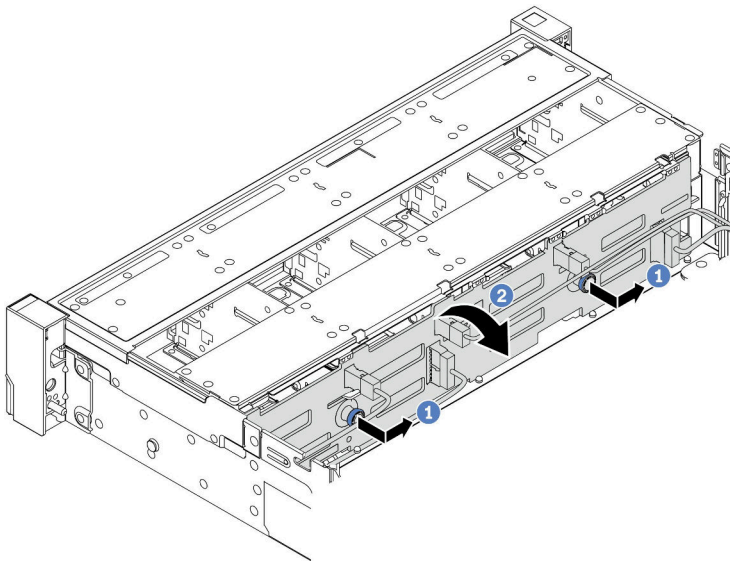
图 87. 卸下 3.5 英寸硬盘背板
