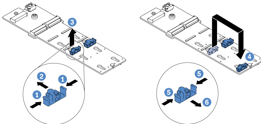
图 140. M.2 固定器调整
