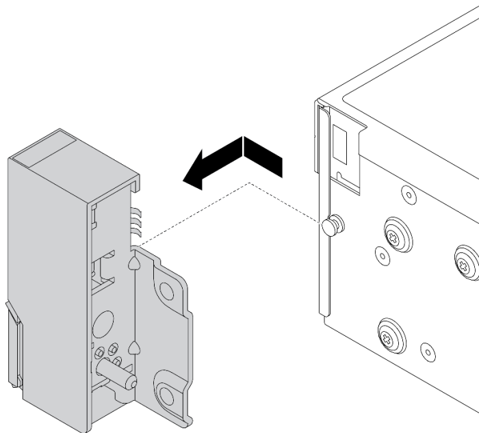
图 156. 卸下机架滑锁
