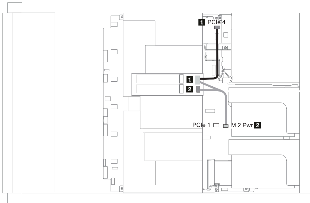
图 21. M.2 cable routing
