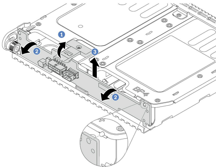
图 89. 卸下 2 x 3.5 英寸硬盘背板
