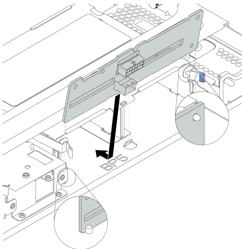
图 85. 安装 4 x 2.5 英寸硬盘背板
