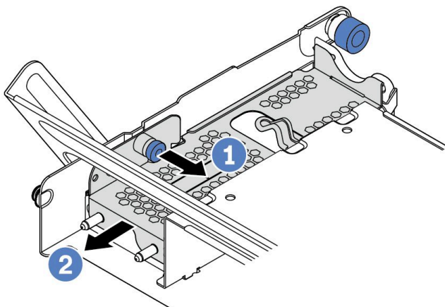
图 170. 卸下金属外盖
