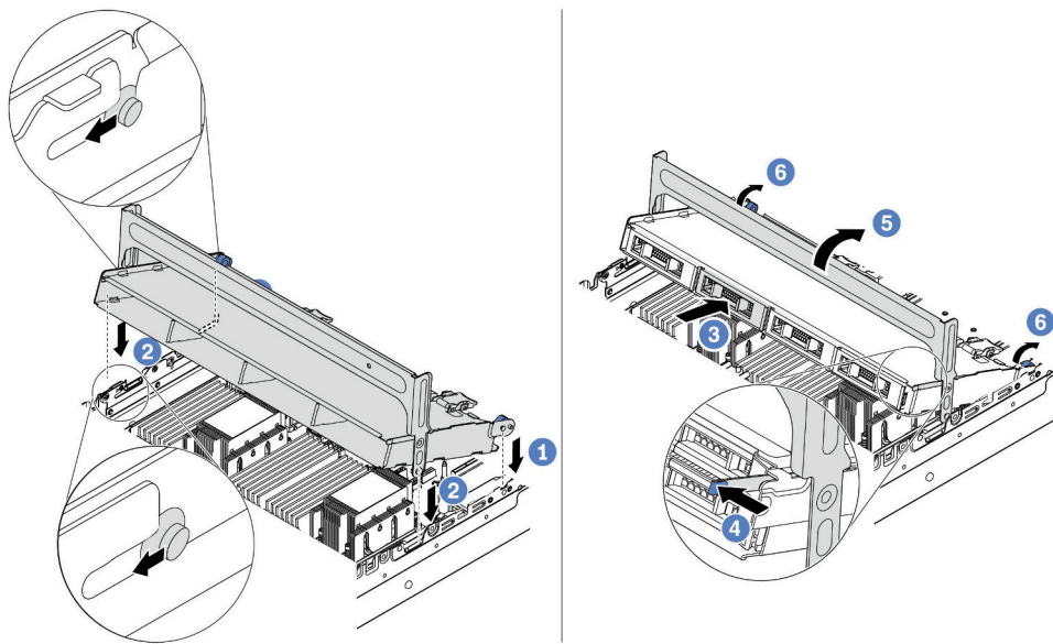
图 106. 安装中间 3.5 英寸硬盘仓和硬盘
