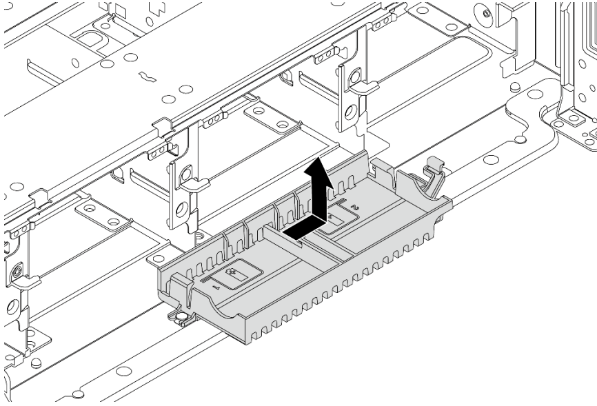
图 173. 卸下超级电容器夹持器
