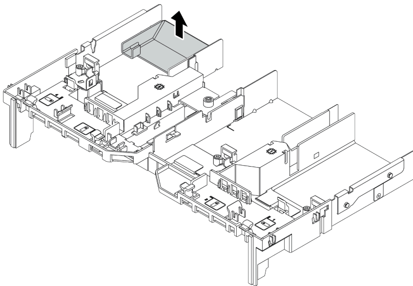
图 71. 卸下附加导风罩
