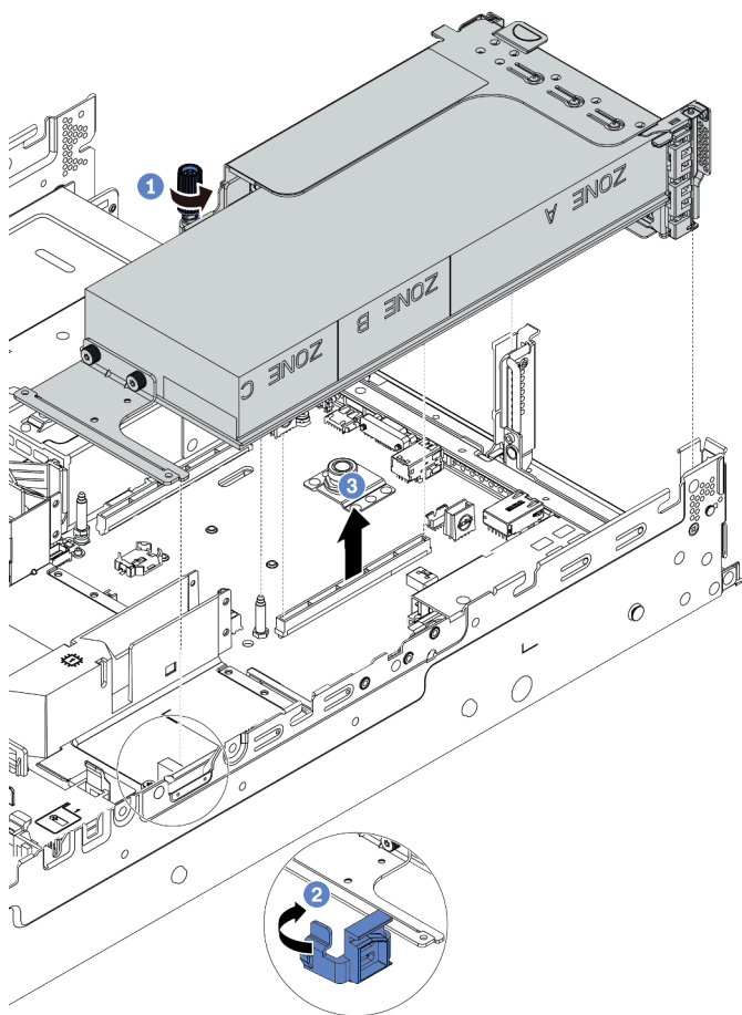
图 69. 卸下转接卡组合件
