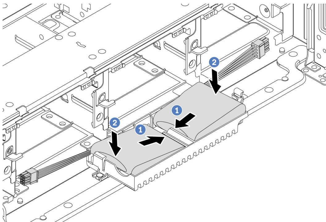
图 175. 安装超级电容器模块
