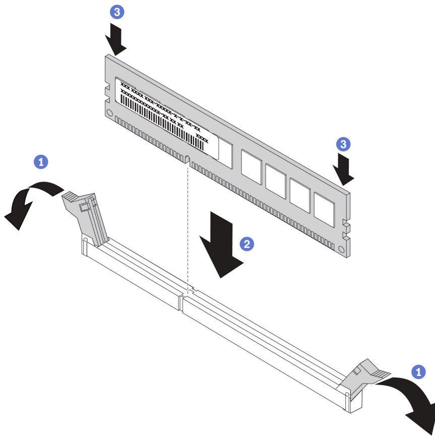
图 147. 安装内存条
