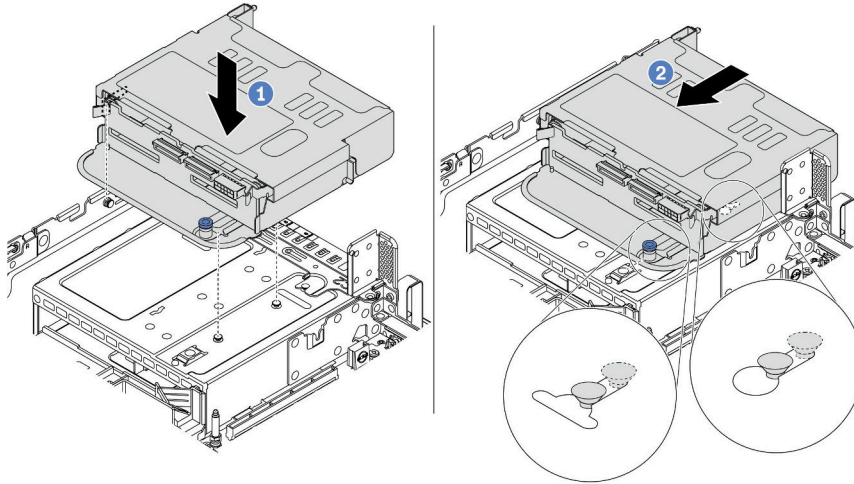
图 113. 安装 4 x 2.5 英寸背面硬盘仓
