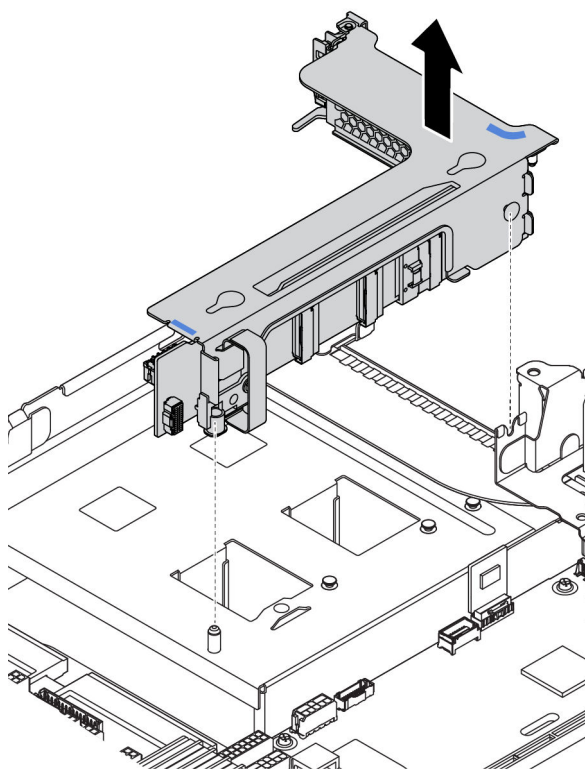
图 184. 卸下转接卡 3 组合件 (双插槽转接卡支架)
