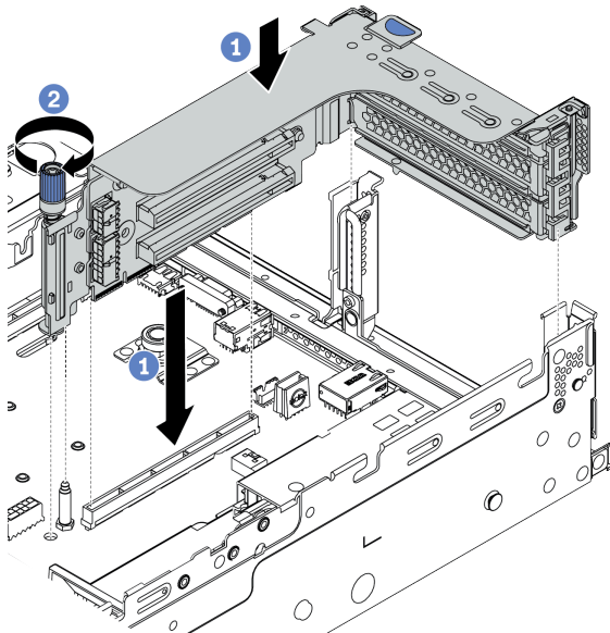
图 191. 转接卡 1/2 组合件安装（三插槽转接卡支架）
