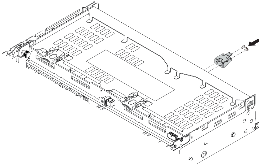
图 111. 安装顶盖支架
