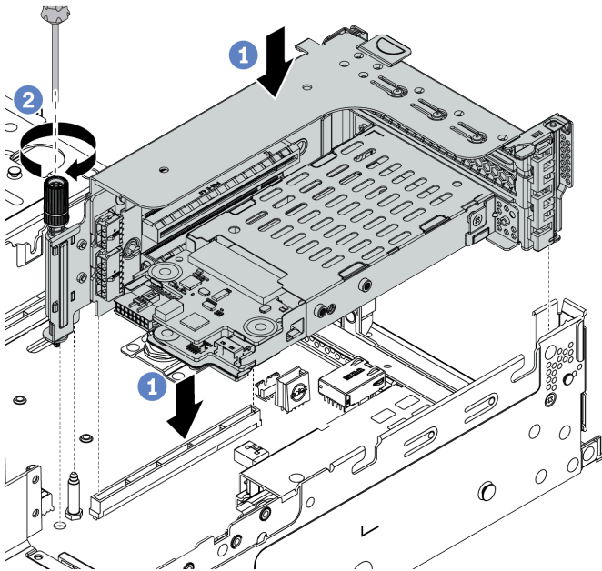
图 122. 安装 7 毫米硬盘仓
