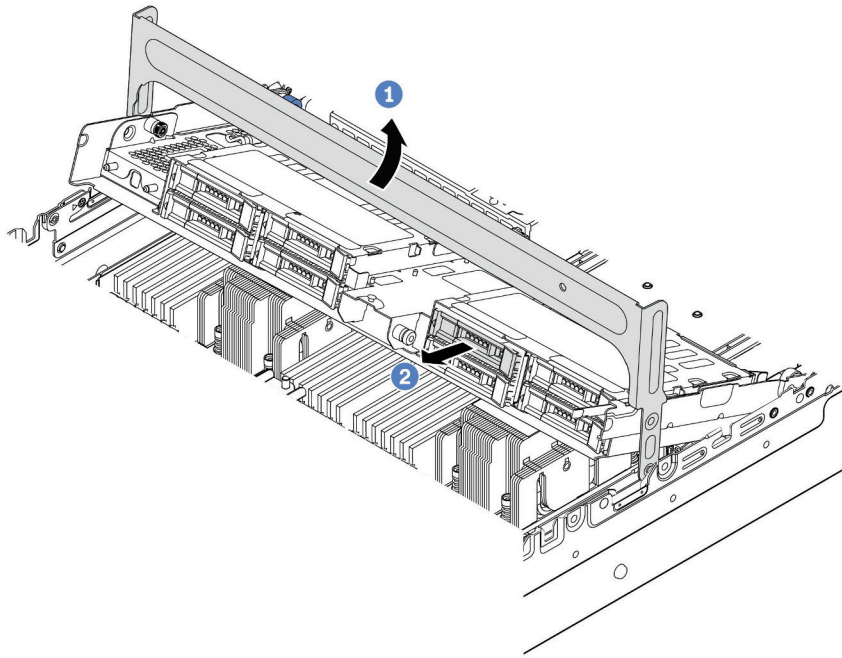
图 97. 打开硬盘仓手柄并卸下硬盘。
