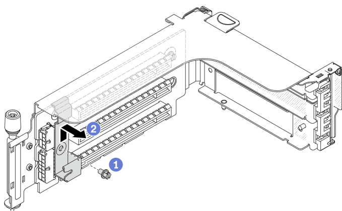
图 118. 卸下 7 毫米硬盘仓固定夹
