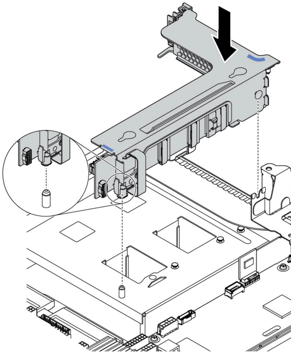
图 193. 转接卡 3 组合件安装
