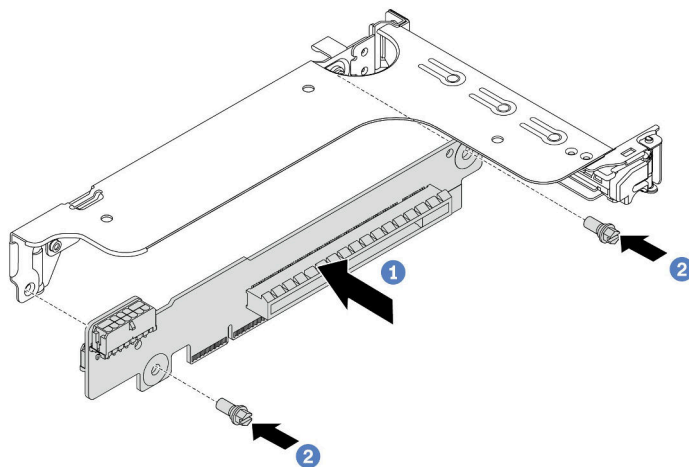
图 189. 转接卡安装（一插槽或两插槽转接卡支架）
