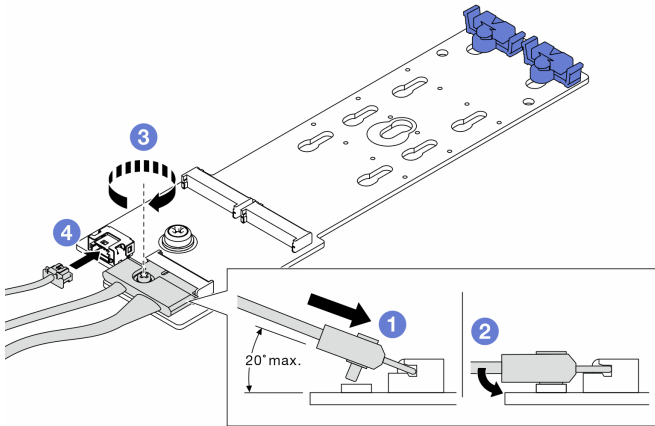
图 144. 连接 M.2 线缆
