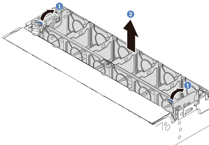
图 204. 卸下系统风扇架
