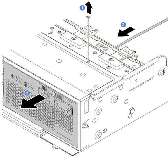
图 65. 卸下正面 I/O 组合件
