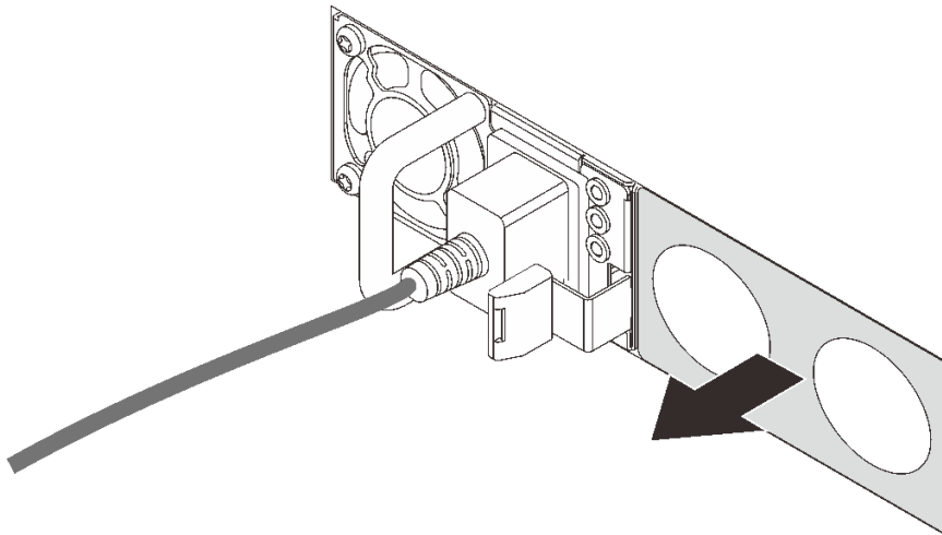
图 127. 卸下热插拔电源模块填充件
