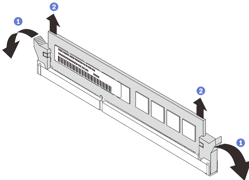
图 145. 卸下内存条
