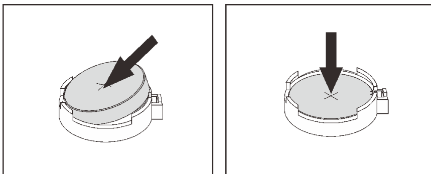
图 61. 安装 CMOS 电池
