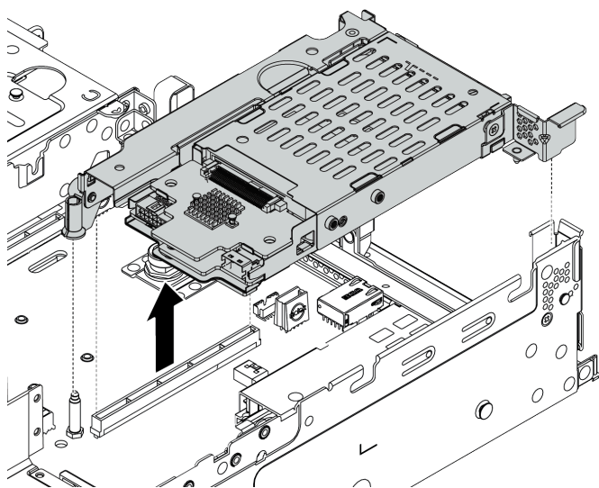
图 119. 卸下转接卡组合件
