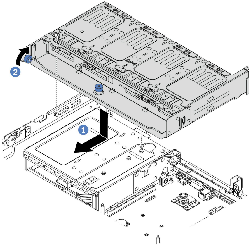
图 115. 安装 8 x 2.5 英寸背面硬盘仓
