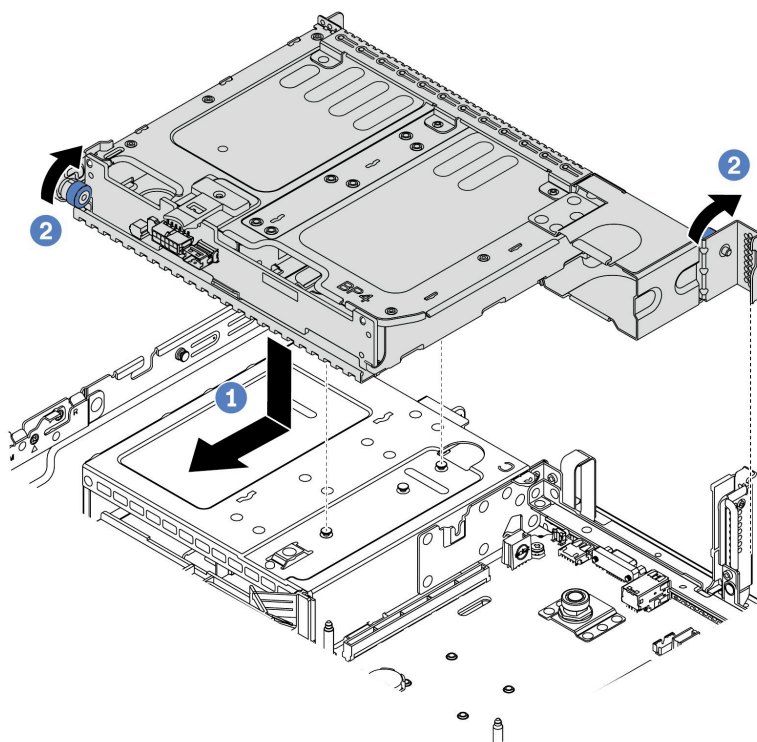
图 108. 安装 2 x 3.5 英寸背面硬盘仓
