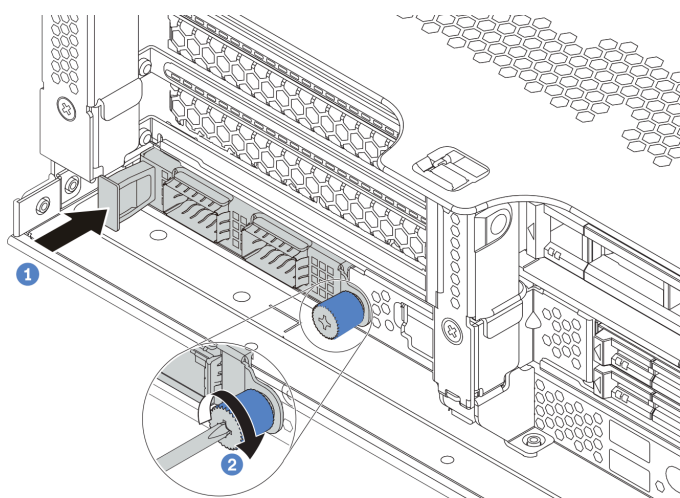
图 149. 安装 OCP 3.0 以太网适配器
