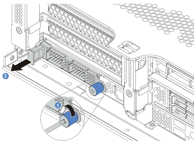
图 148. 卸下 OCP 3.0 以太网适配器
