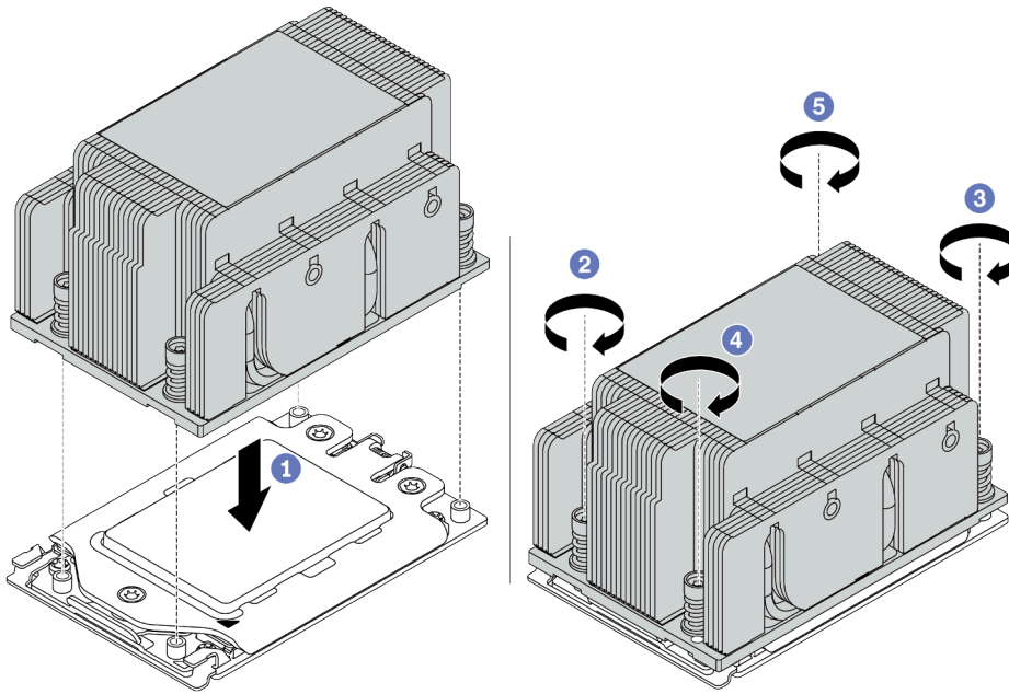
图 215. 安装标准散热器
