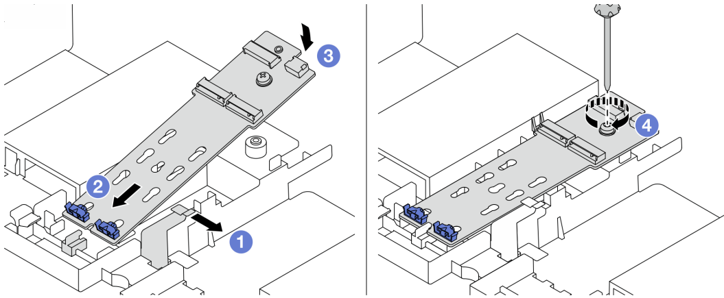
图 142. M.2 适配器安装
