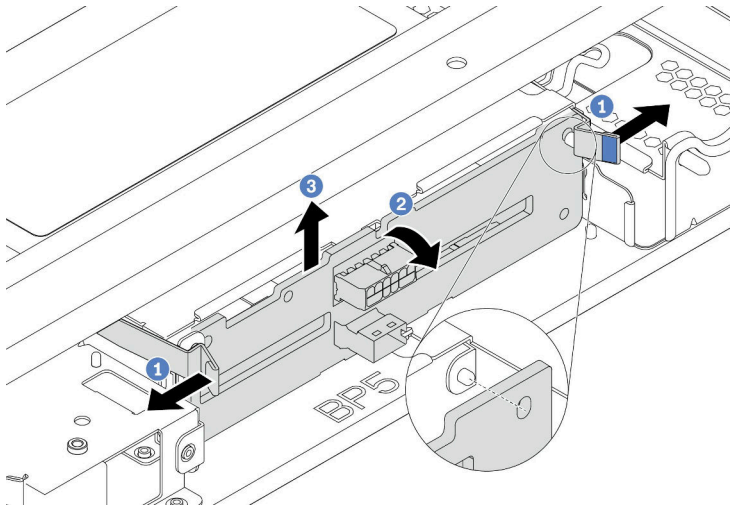
图 83. 卸下 4 x 2.5 英寸硬盘背板
