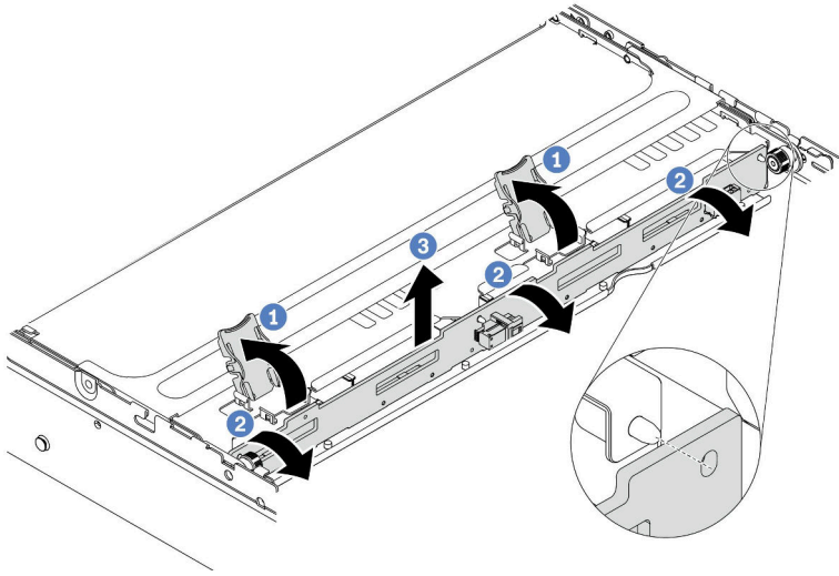
图 90. 卸下 4 x 3.5 英寸硬盘背板
