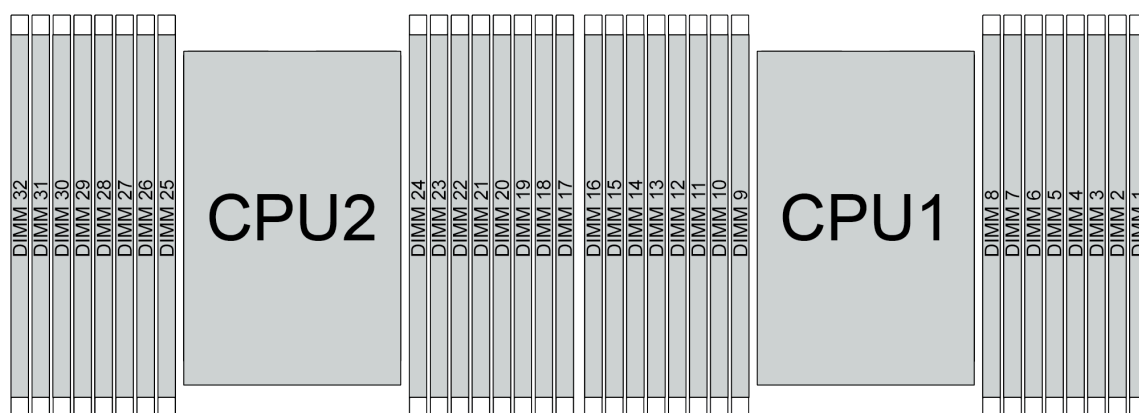
图 146. 内存条位置
