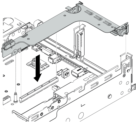
图 192. 转接卡 1/2 组合件安装 (单插槽转接卡支架)
