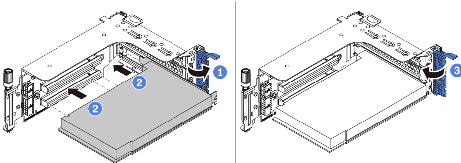
图 190. 安装 PCIe 适配器
