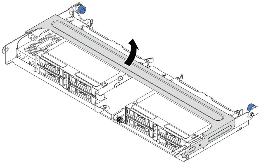
图 167. 打开中间硬盘仓的手柄
