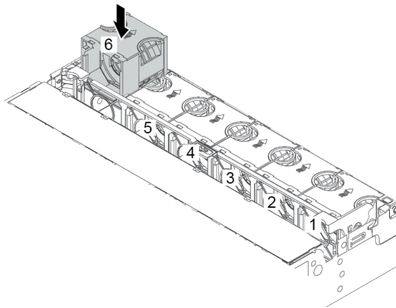
图 203. 安装系统风扇
