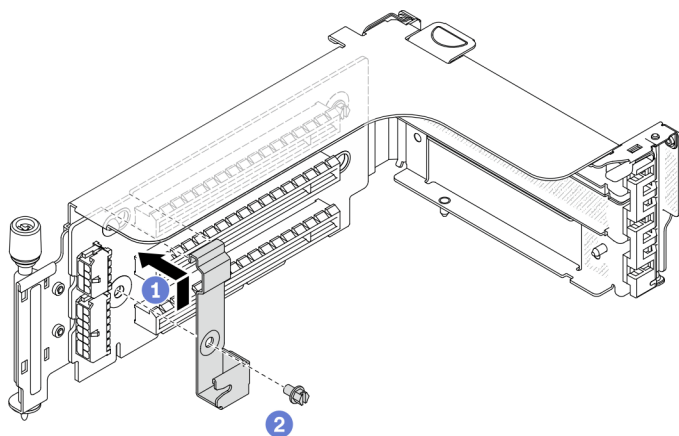
图 120. 安装 7 毫米硬盘仓固定夹
