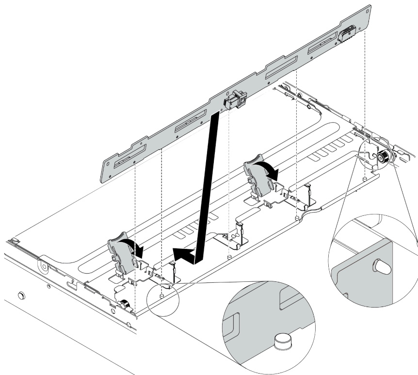
图 92. 安装 4 x 3.5 英寸硬盘背板
