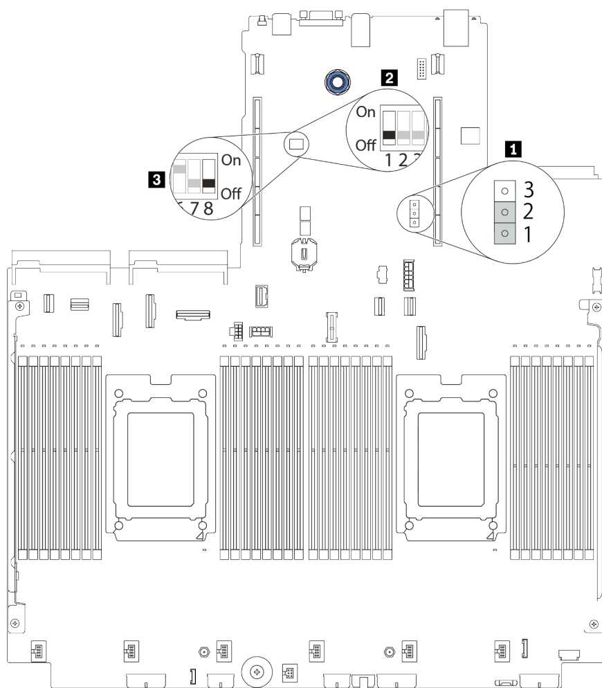
图 13. 主板上的开关组和跳线位置
