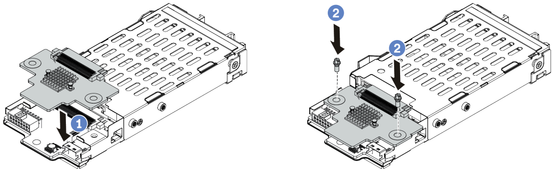
图 96. 安装 7 毫米硬盘背板 (顶部)
