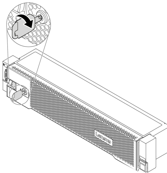
图 197. 解锁安全挡板
