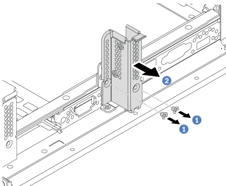
图 178. 卸下 B1 后壁支架
