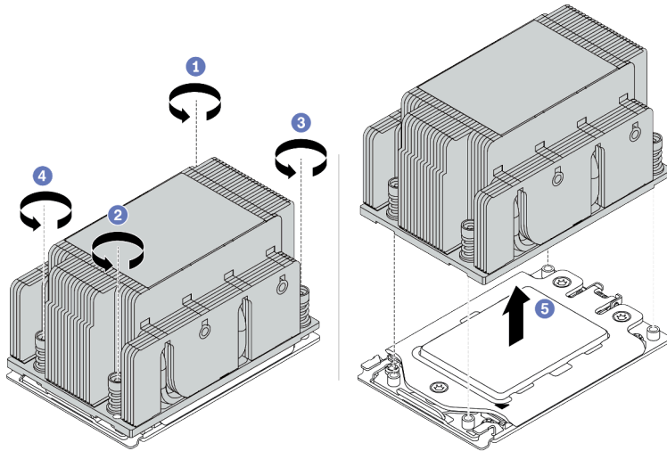
图 210. 卸下标准散热器
