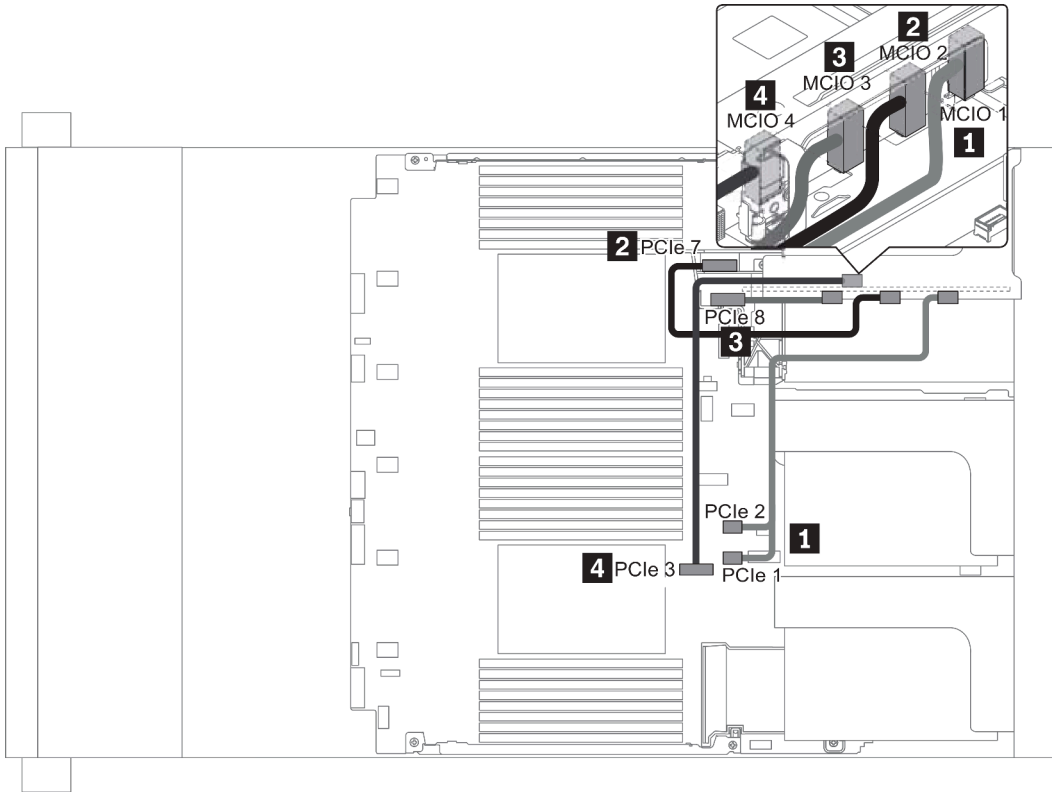
图 17. 转接卡 3 (x8/x8 或 x16/x16 PCIe) 的线缆布放
