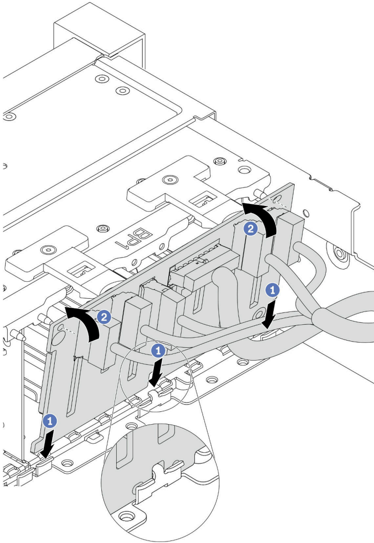
图 82. 安装 2.5 英寸硬盘背板
