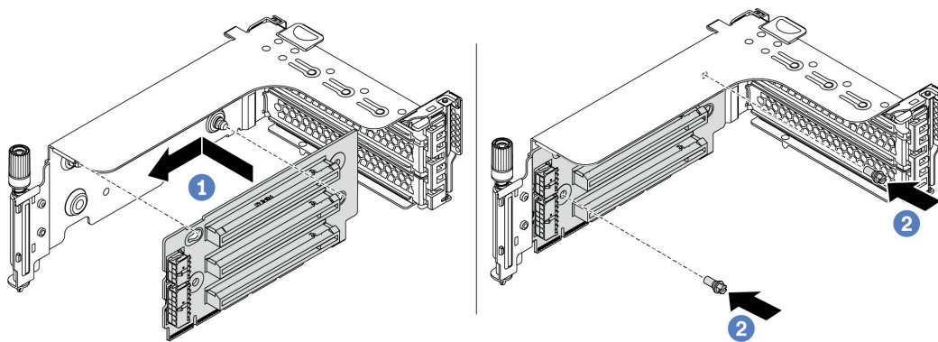
图 188. 转接卡安装（三插槽转接卡支架）
