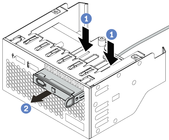
图 66. 卸下 LCD 诊断程序面板
