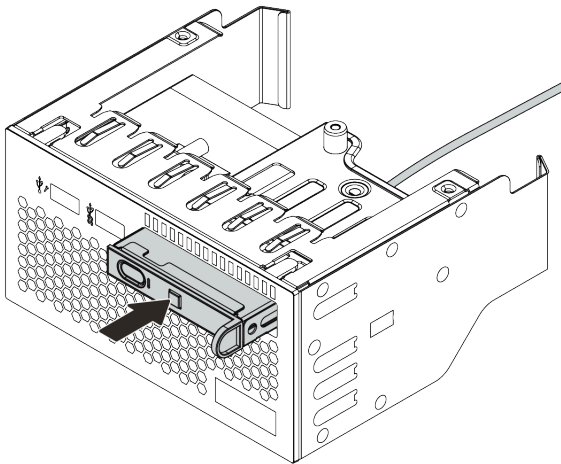
图 68. 安装 LCD 诊断面板
