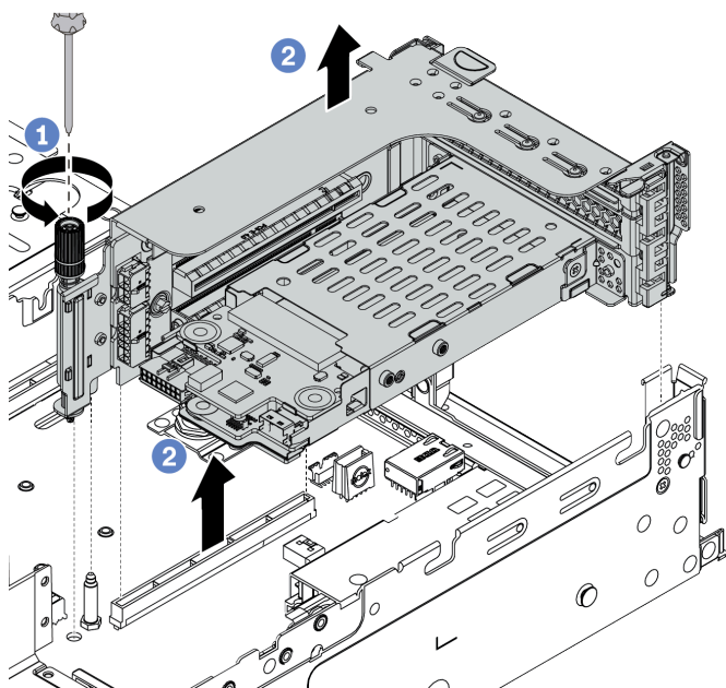
图 116. 卸下转接卡组合件
