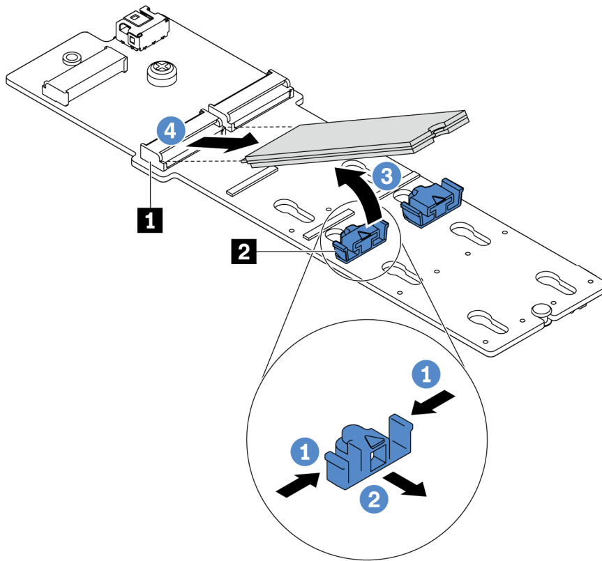
图 138. 卸下 M.2 硬盘
