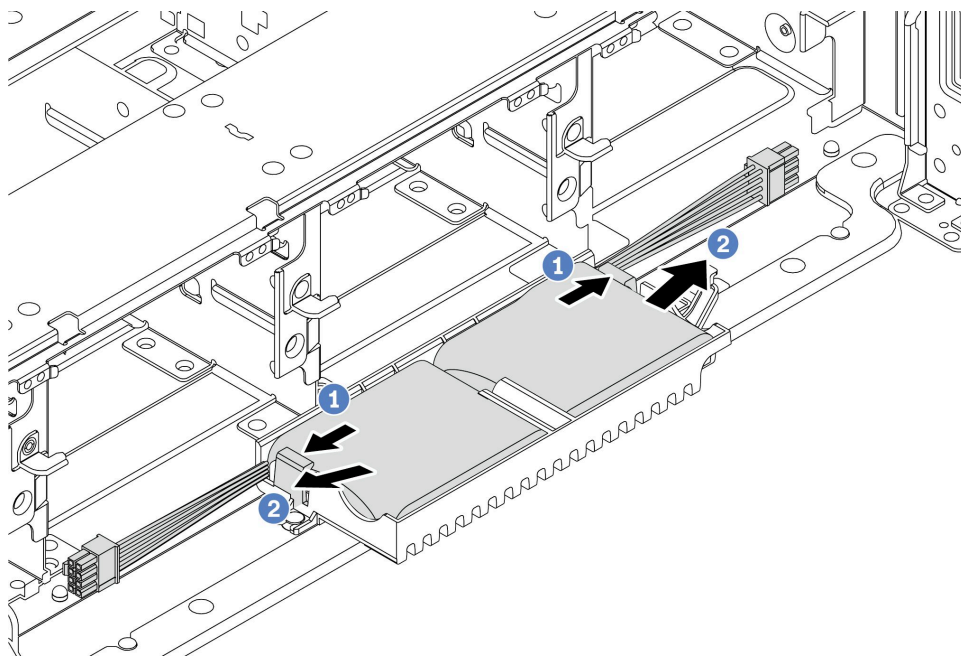
图 172. 卸下超级电容器模块
