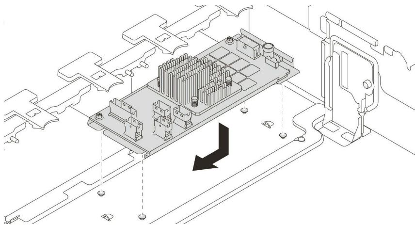
图 130. 安装内部 CFF RAID/HBA 适配器
