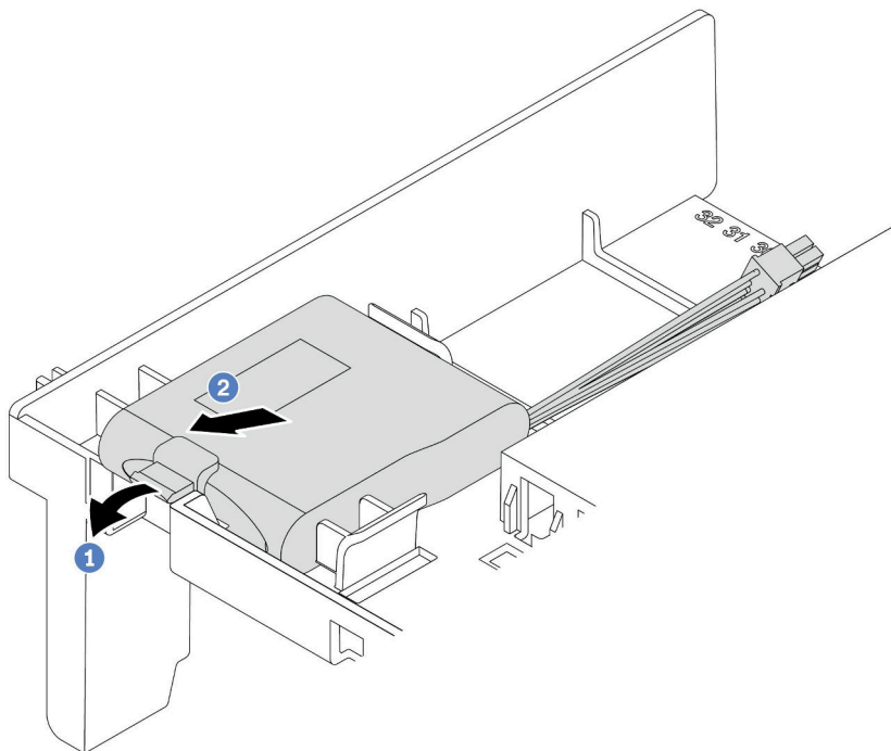
图 165. 卸下超级电容器模块
