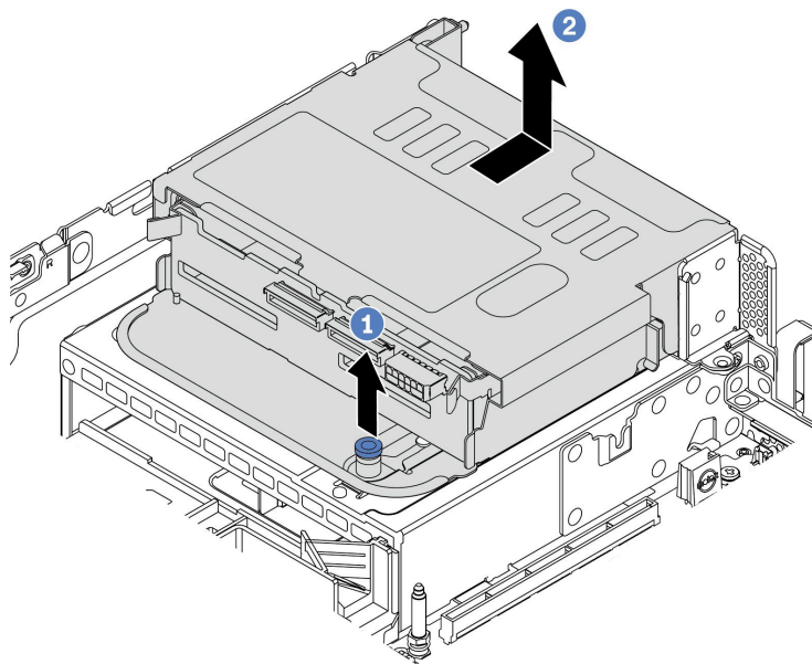
图 112. 卸下 4 x 2.5 英寸背面硬盘仓
