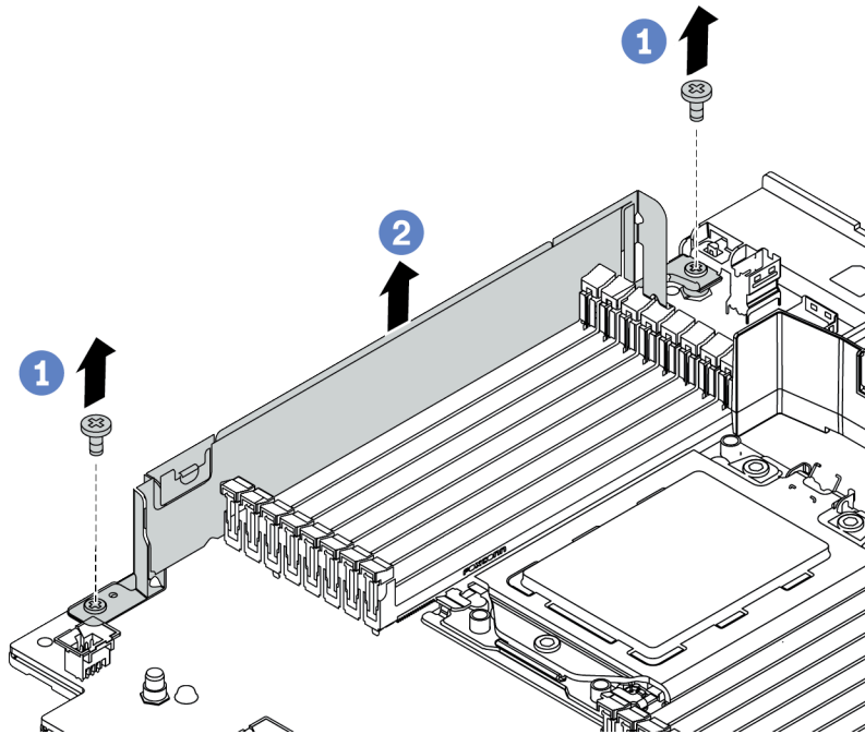
图 58. 卸下线缆固定扣
