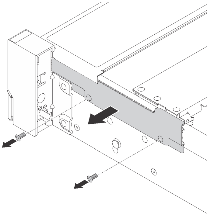
图 154. 卸下线缆固定器
