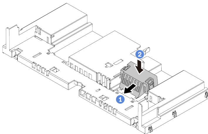
图 56. 将填充件安装到标准导风罩
