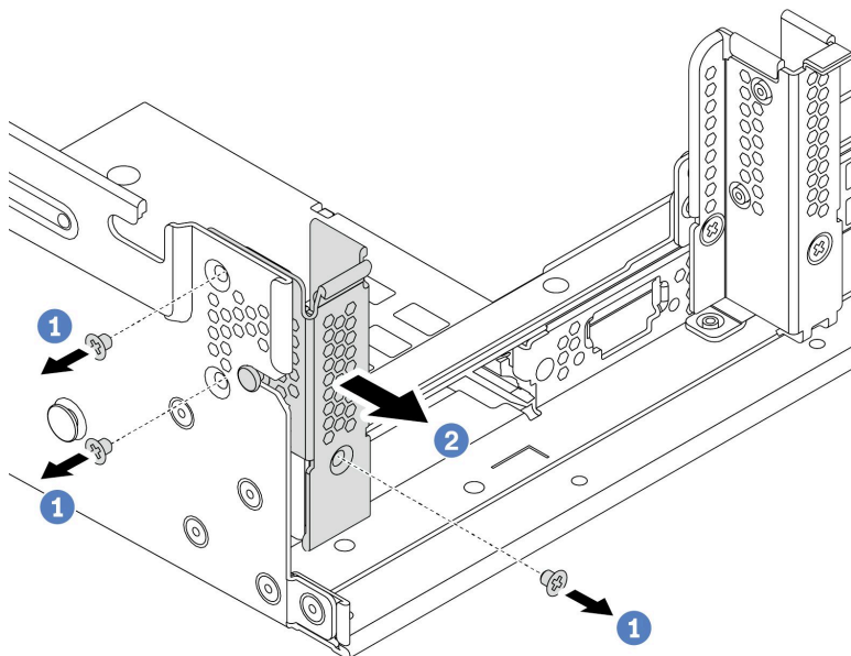
图 176. A1 背面壁挂支架安装
