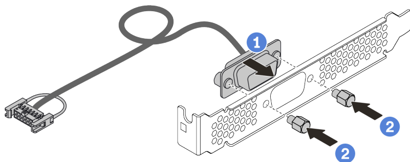
图 196. 组装串口模块
