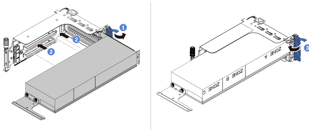
图 74. 将 GPU 适配器安装到转接卡架中
