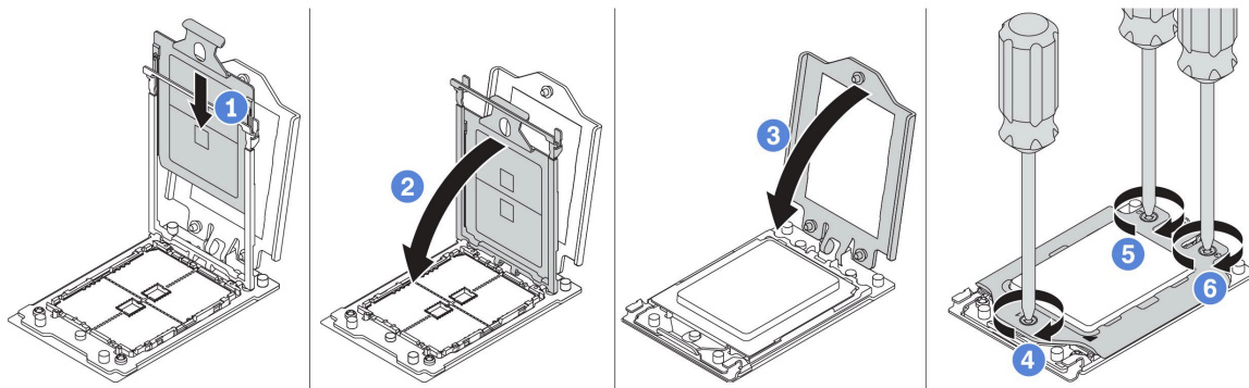
图 213. 安装处理器
