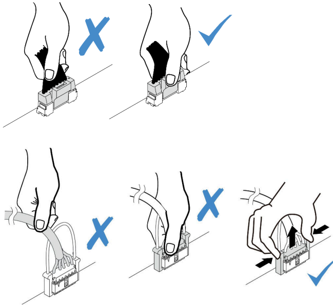
图 64. 拔下正面 I/O 组合件线缆
