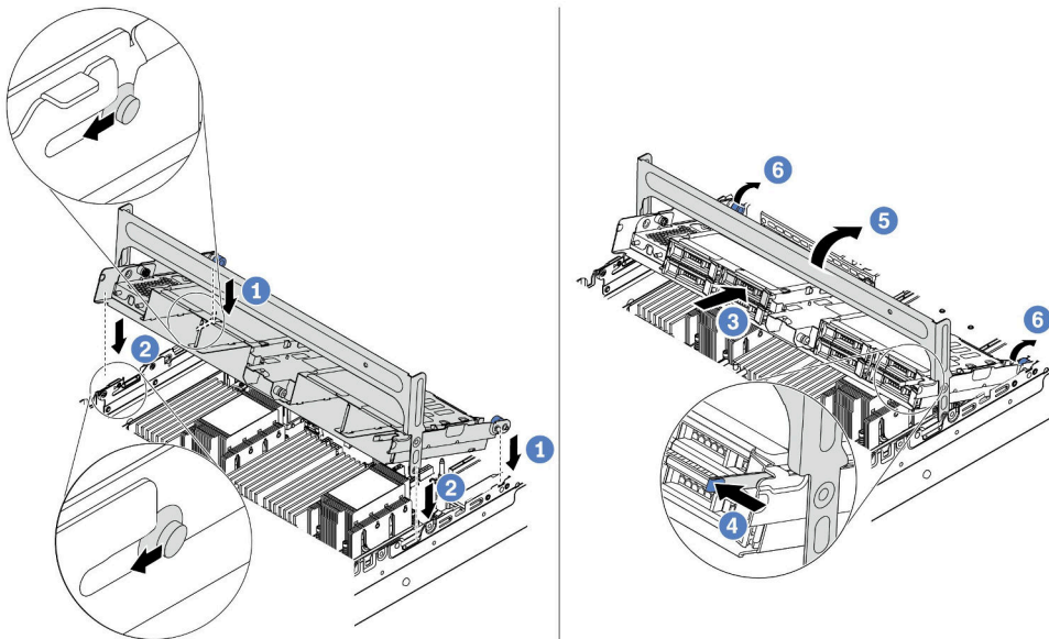
图 101. 安装中间 2.5 英寸硬盘仓和硬盘
