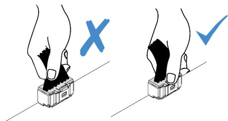
图 136. 拔下 M.2 线缆
