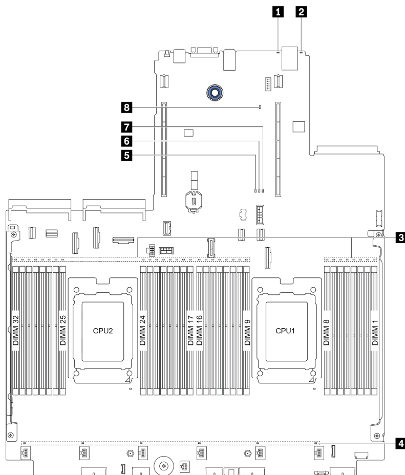
图 12. 主板 LED
