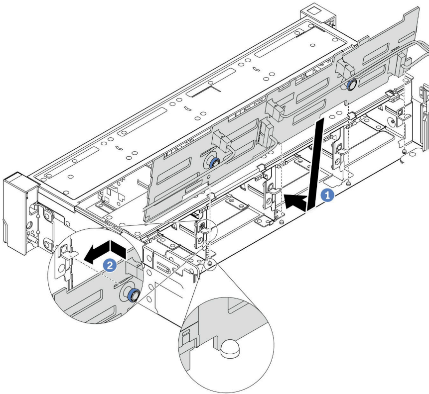
图 88. 安装 3.5 英寸硬盘背板
