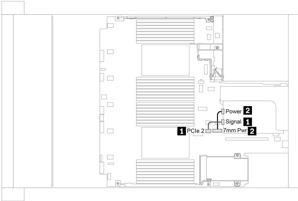
图 20. 7mm 电缆路由当安装一个处理器
