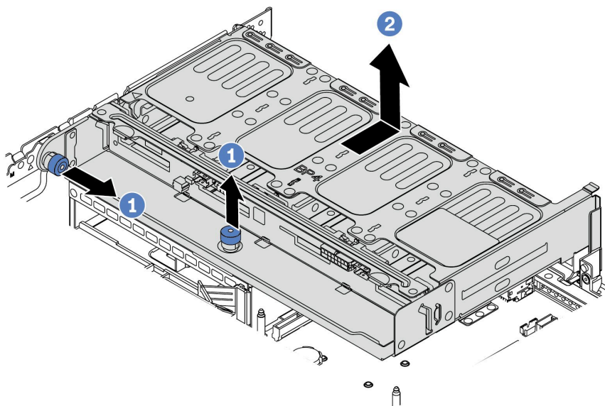
图 114. 卸下 8 x 2.5 英寸背面硬盘仓
