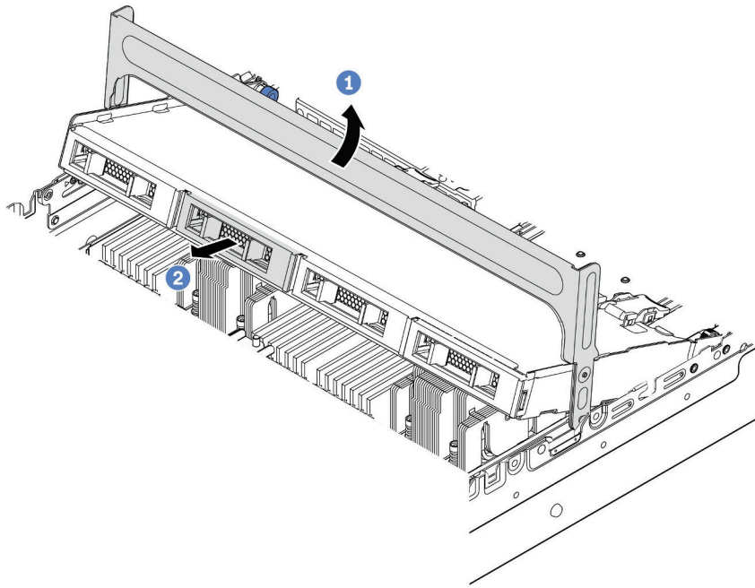
图 102. 打开硬盘仓手柄并卸下硬盘。
