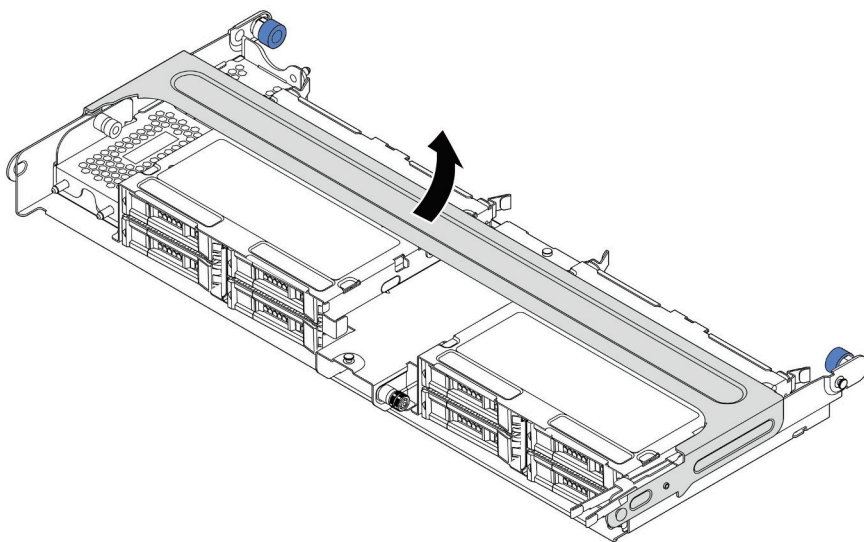
图 169. 打开中间硬盘仓的手柄
