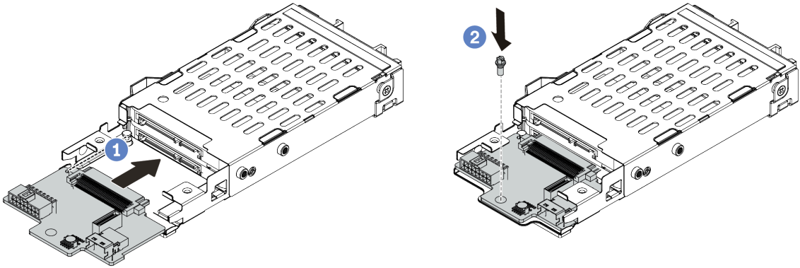
图 95. 安装 7 毫米硬盘背板 (底部)
