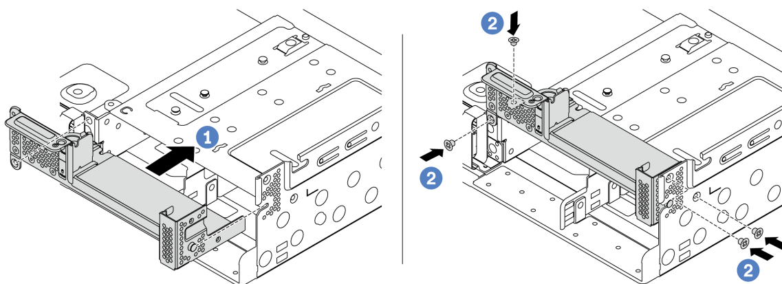
图 181. C1 背面壁挂支架安装
