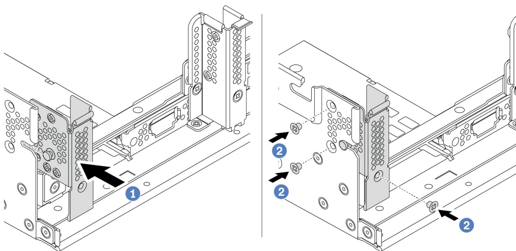
图 177. A1 背面壁挂支架安装
