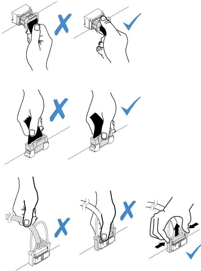
图 153. 拔下 VGA 和正面 I/O 组合件线缆
