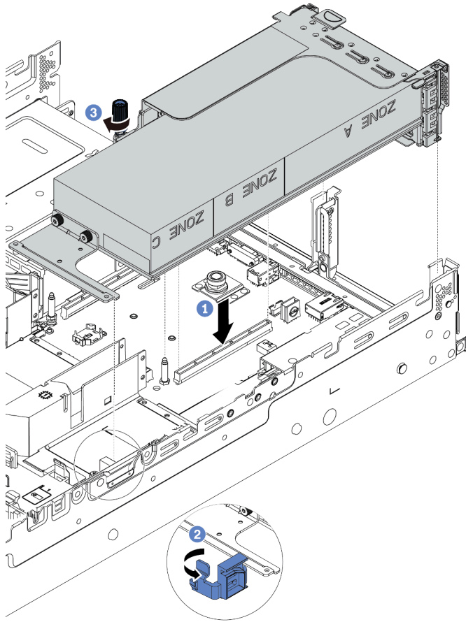
图 75. 安装转接卡组合件
