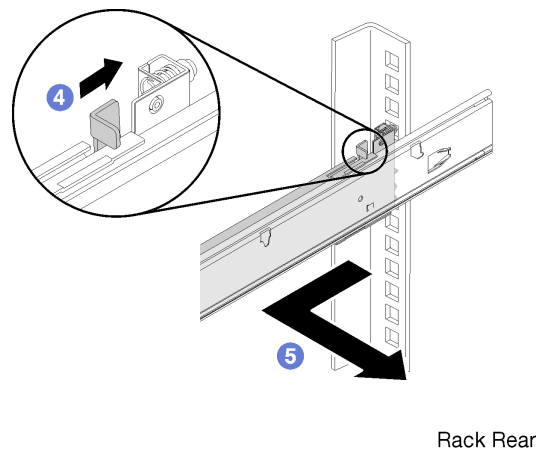
Рис. 23. Снятие левой направляющей сзади
