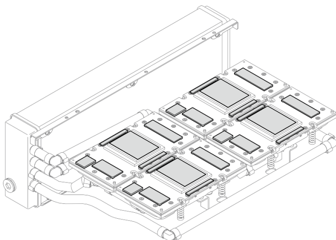
Figura 238. Limpieza del PCM y las almohadillas de masilla de las placas de frío
