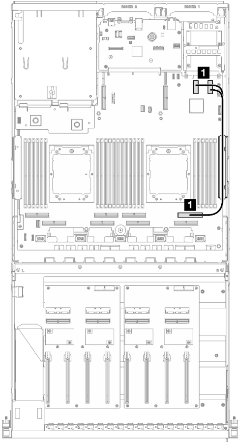
Figura 329. Disposición de los cables del módulo de OCP
