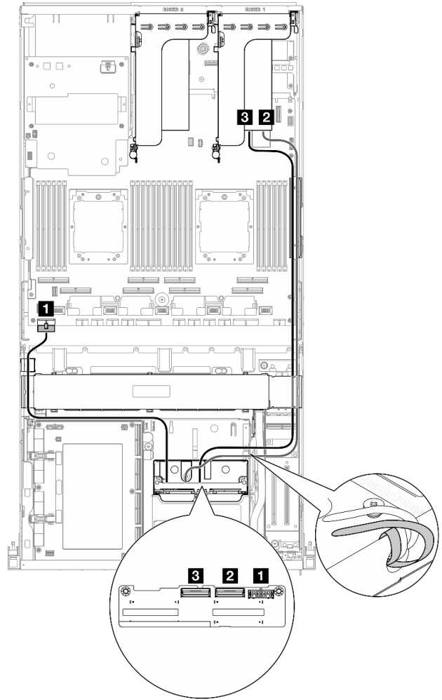
Figura 341. Disposición de los cables de la placa posterior de la unidad de 2,5 pulgadas (adaptador RAID en la expansión PCIe 1)
