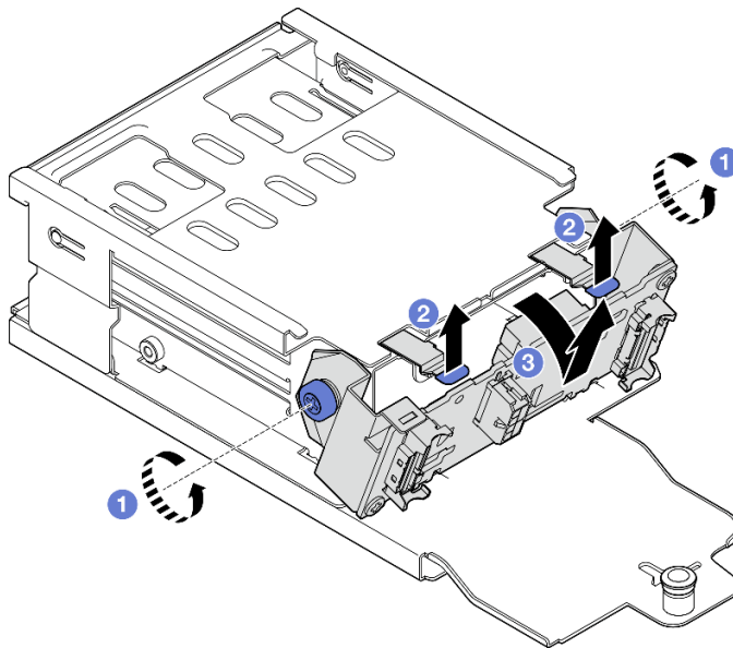
Figura 130. Extracción del módulo de la placa posterior de la unidad E3.S
