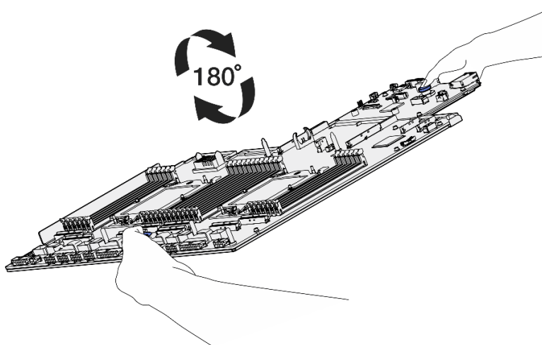
Figura 94. Giro del conjunto de la placa del sistema
