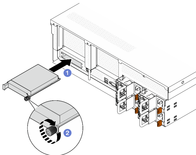
Figura 60. Instalación del módulo de OCP
