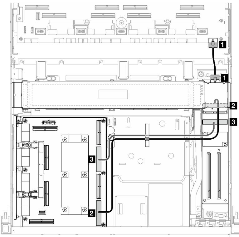
Figura 358. Disposición de los cables de la placa de expansión de E/S frontal
