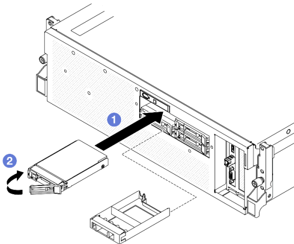
Figura 162. Instalación de unidad de intercambio en caliente de 2,5 pulgadas
