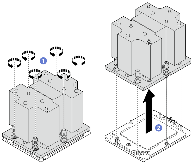
Figura 81. Extracción del disipador de calor
