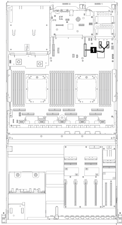
Figura 313. Disposición de los cables del módulo de OCP
