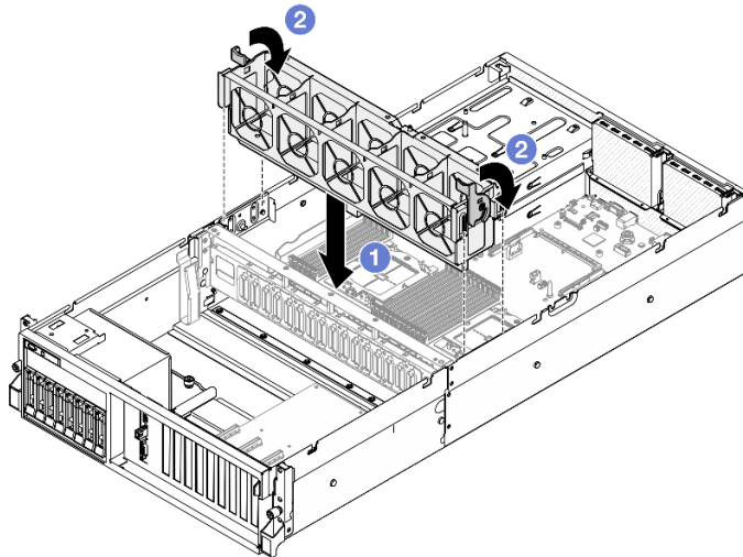
Figura 22. Instalación de la caja del ventilador
