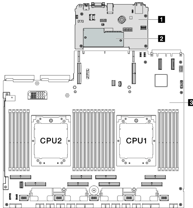
Figura 88. Disposición del conjunto de la placa del sistema
