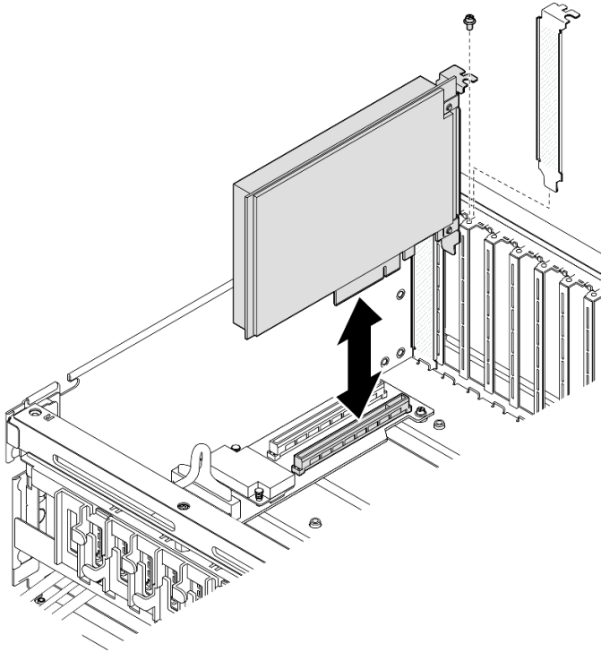
Figura 63. Instalación del adaptador PCIe frontal
