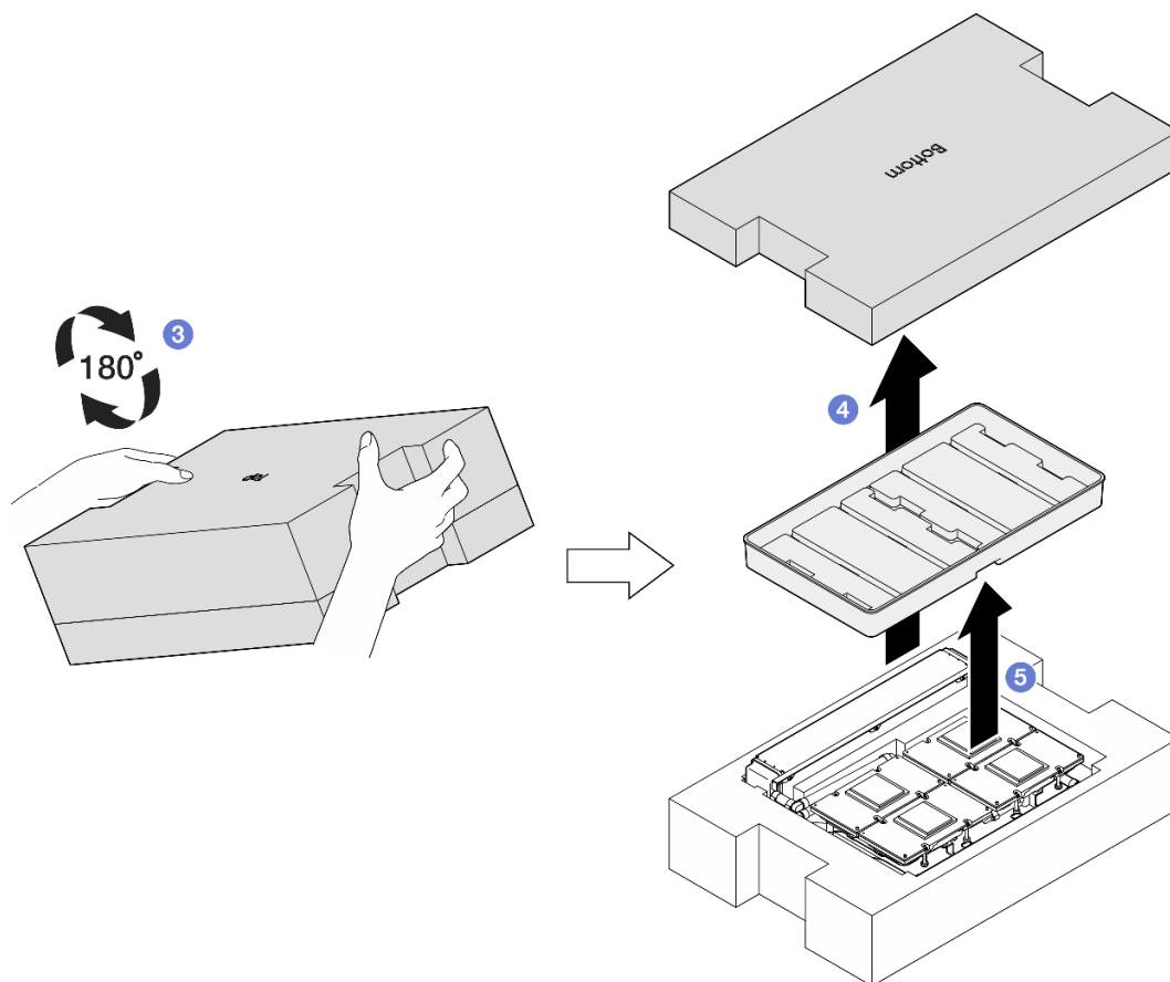
Figura 237. Volteo del L2A hacia abajo
