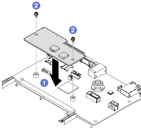
Figura 90. Instalación del Firmware y módulo de seguridad de RoT
