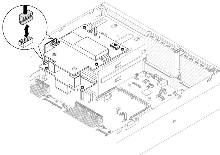
Figura 276. Conexión del cable de banda lateral
