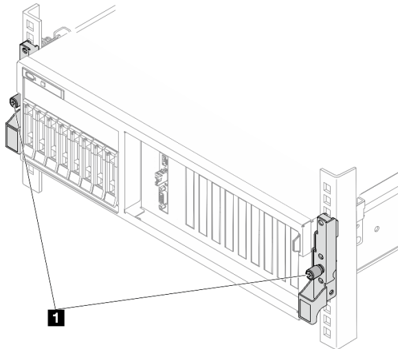
Figura 2. Desenganche del servidor del bastidor
