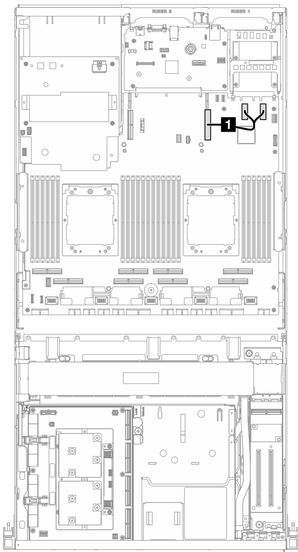
Figura 367. Disposición de los cables del módulo de OCP
