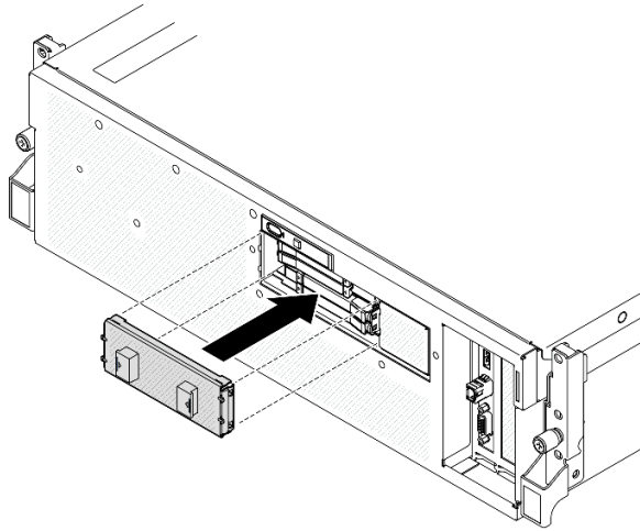
Figura 185. Instalación de la cubierta del compartimiento de la unidad E3.S
