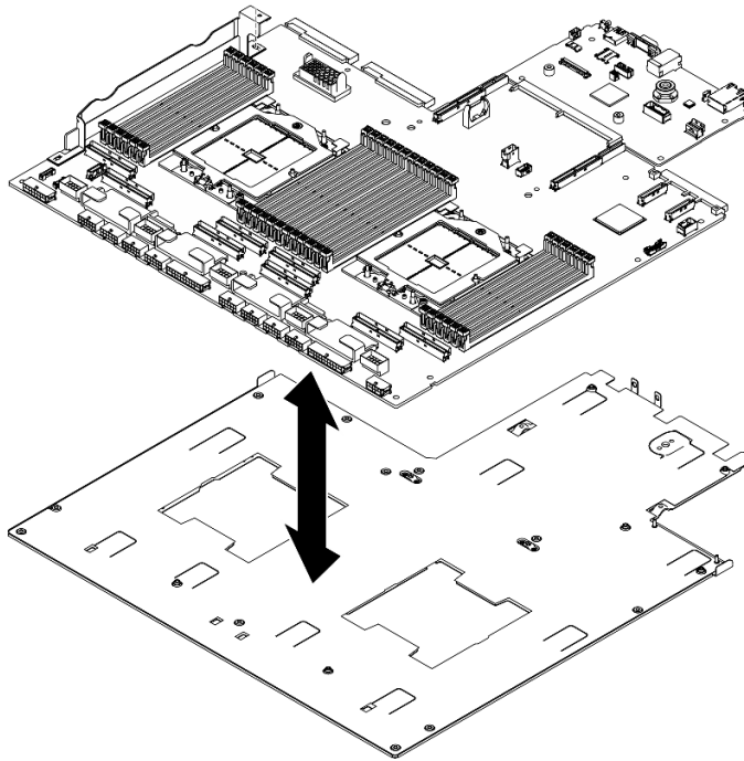
Figura 98. Desensamblaje del conjunto de la placa del sistema
