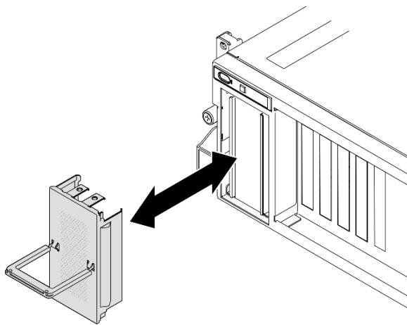
Figura 127. Instalación de la cubierta del compartimiento de la unidad EDSFF
