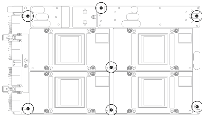
Figura 268. Instalación del tornillo Phillips n.º 1
