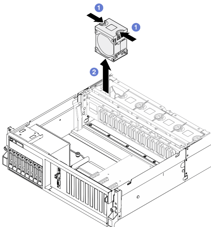
Figura 19. Extracción del ventilador
