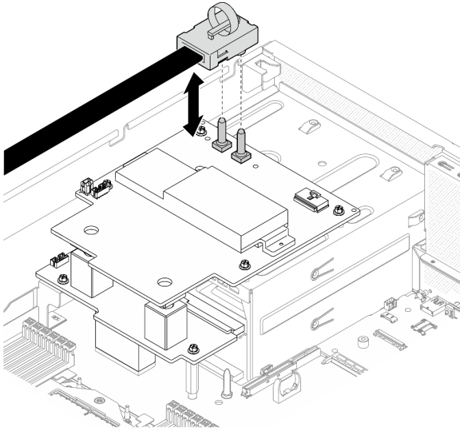
Figura 271. Desconexión del cable de alimentación del Conjunto de placa de GPU SXM5
