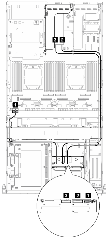
Figura 340. Disposición de los cables de la placa posterior de la unidad de 2,5 pulgadas (adaptador RAID en la expansión PCIe 2)
