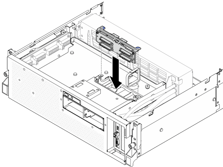
Figura 165. Instalación del módulo de la placa posterior de la unidad de 2,5 pulgadas
