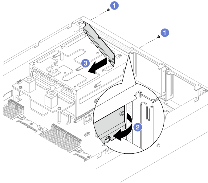
Figura 158. Extracción del deflector posterior de flujo de aire térmico
