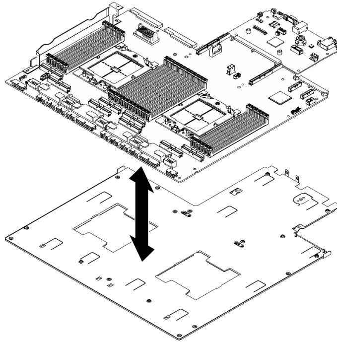
Figura 101. Instalación del conjunto de la placa del sistema
