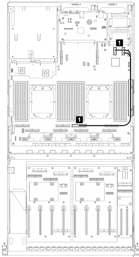
Figura 332. Disposición de los cables del módulo de OCP
