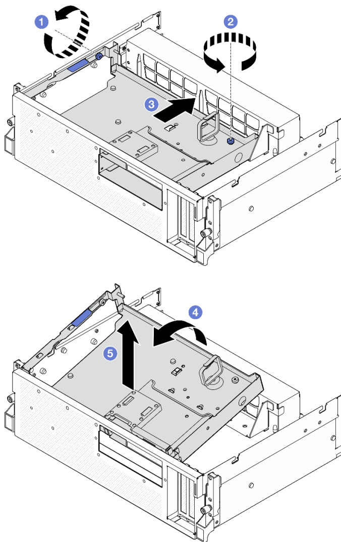
Figura 197. Extracción de la bandeja de unidades frontal
