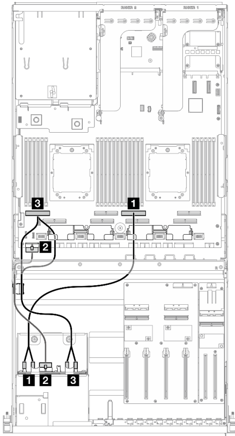
Figura 299. Disposición de los cables de la placa posterior de unidad de 2,5 pulgadas
