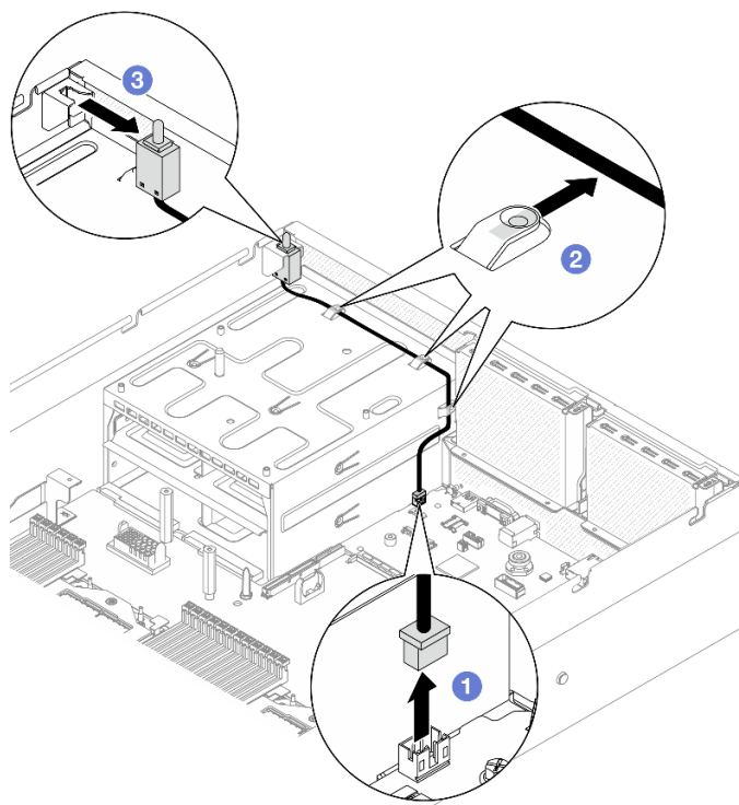
Figura 36. Extracción del conmutador de intrusión
