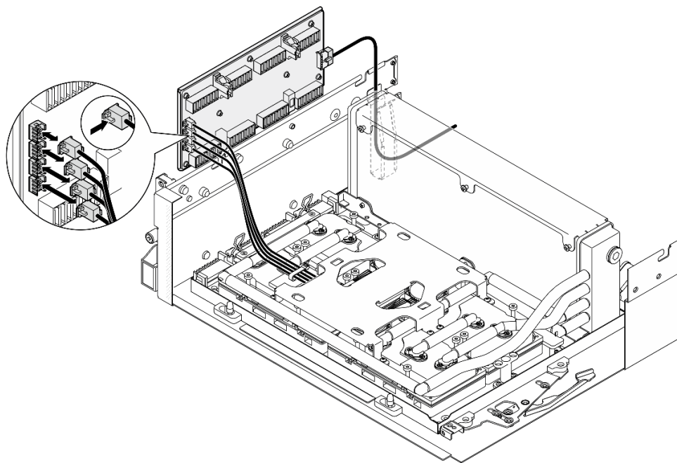
Figura 224. Conexión del cable de la bomba del conjunto de la placa de frío
