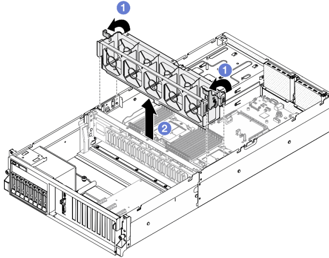
Figura 21. Extracción de la caja del ventilador
