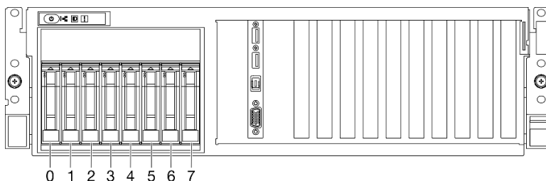
Figura 112. Numeración de la bahía de unidad de 2,5 pulgadas en el Modelo de GPU 4-DW
