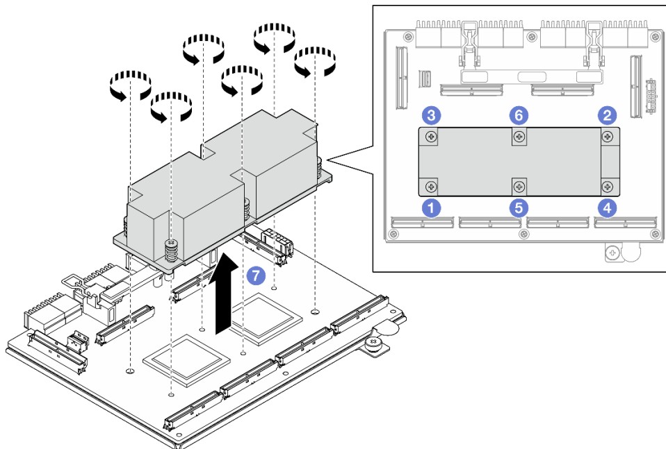
Figura 280. Extracción del disipador de calor de la Placa de conmutador PCIe de SXM5
