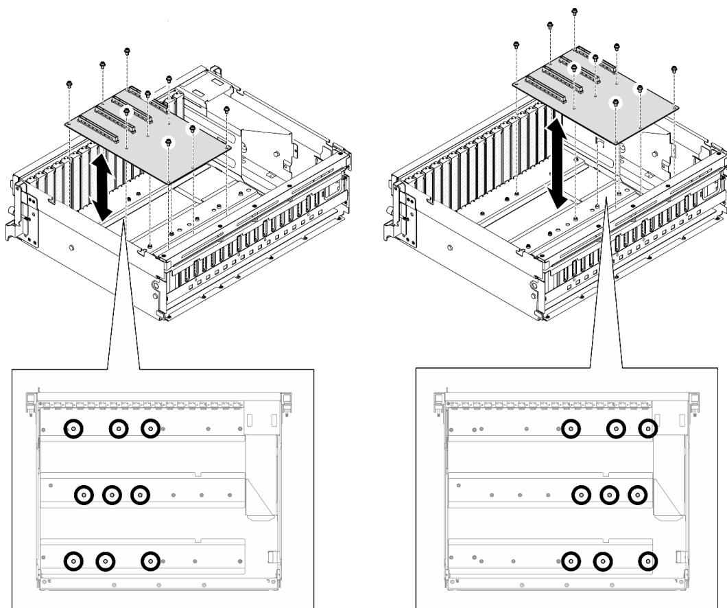
Figura 150. Instalación de una placa de distribución de GPU: Modelo de GPU 8-DW
