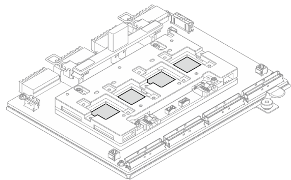
Figura 178. Limpieza de las almohadillas de masilla del ASIC
