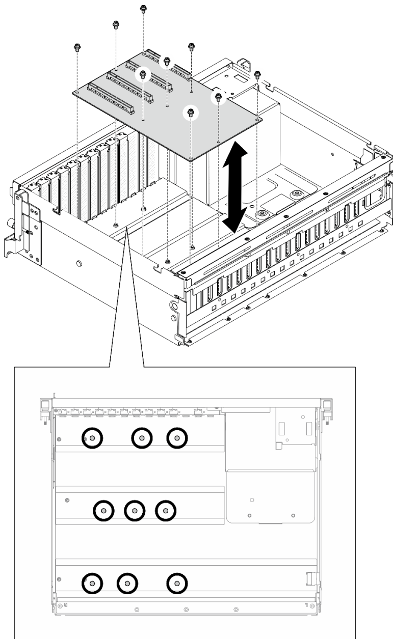
Figura 147. Extracción de la placa de distribución de GPU: Modelo de GPU 4-DW
