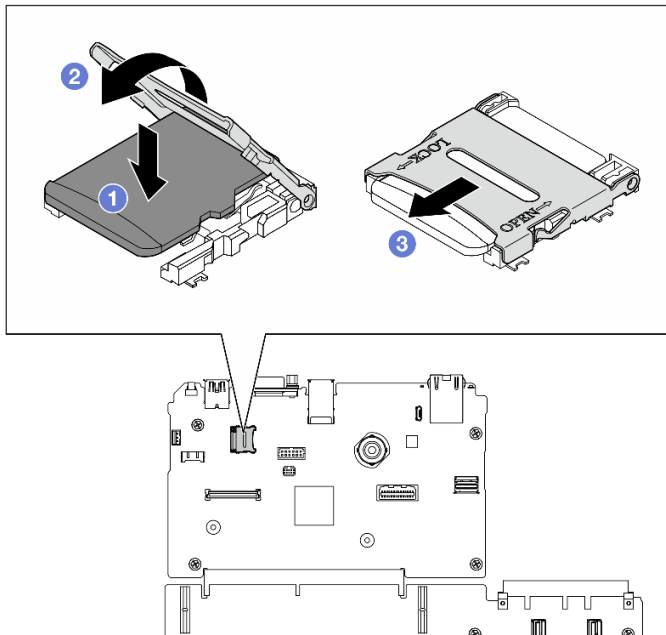
Figura 54. Tarjeta microSD, instalación
