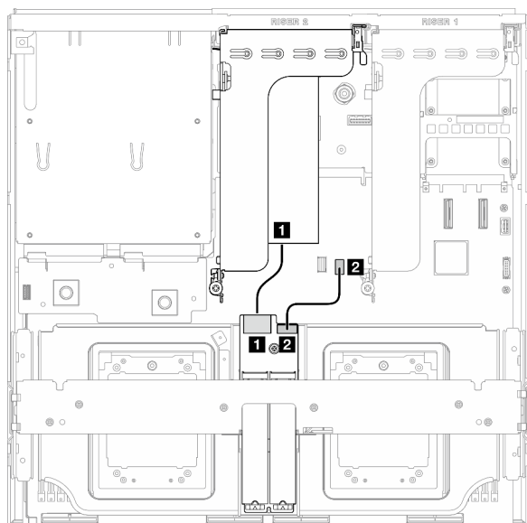
Figura 327. Disposición de los cables para la placa posterior M.2 SATA/x4 NVMe (adaptador RAID en la expansión de PCIe 2)
