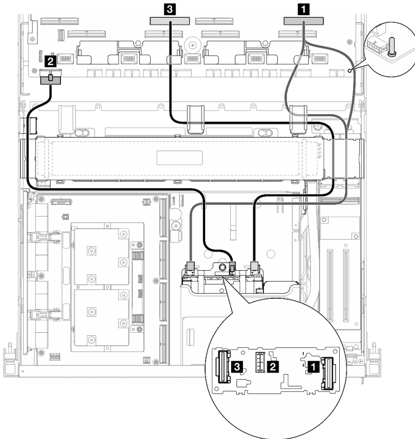
Figura 356. Disposición de los cables de la placa posterior de unidad E3.S
