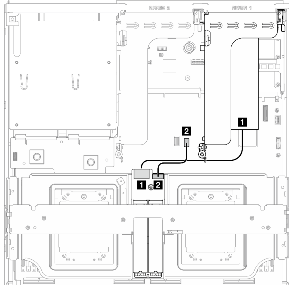
Figura 363. Disposición de los cables para la placa posterior M.2 SATA/x4 NVMe (adaptador RAID en la expansión de PCIe 1)
