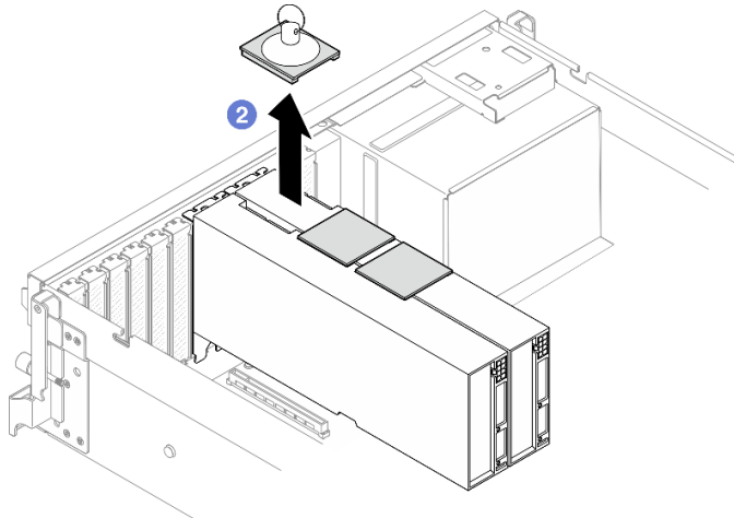
Figura 153. Extracción del Puente de enlace del adaptador de GPU
