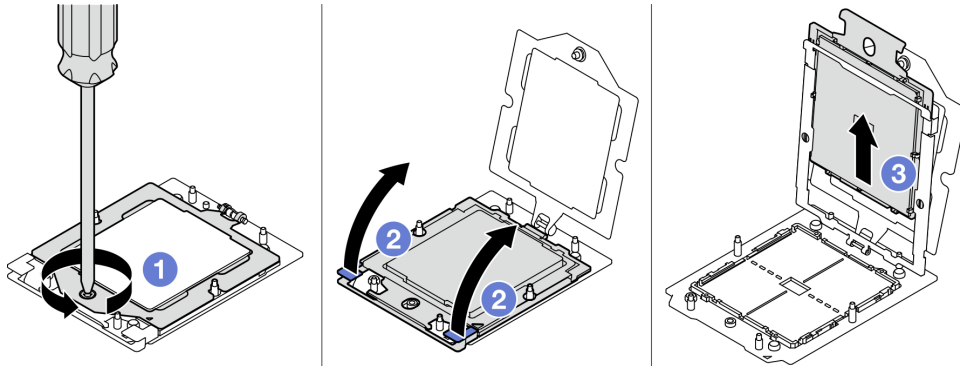
Figura 82. Extracción de un procesador
