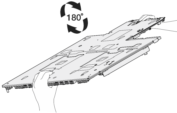
Figura 96. Giro del conjunto de la placa del sistema
