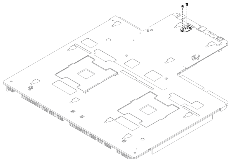
Figura 104. Instalación del tornillo
