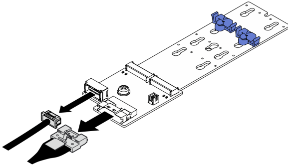
Figura 42. Desconexión de cable de la placa posterior SATA/x4 NVMe M.2
