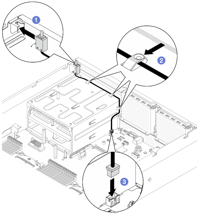
Figura 37. Instalación del conmutador de intrusión
