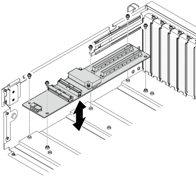
Figura 140. Instalación de la placa de expansión de E/S frontal
