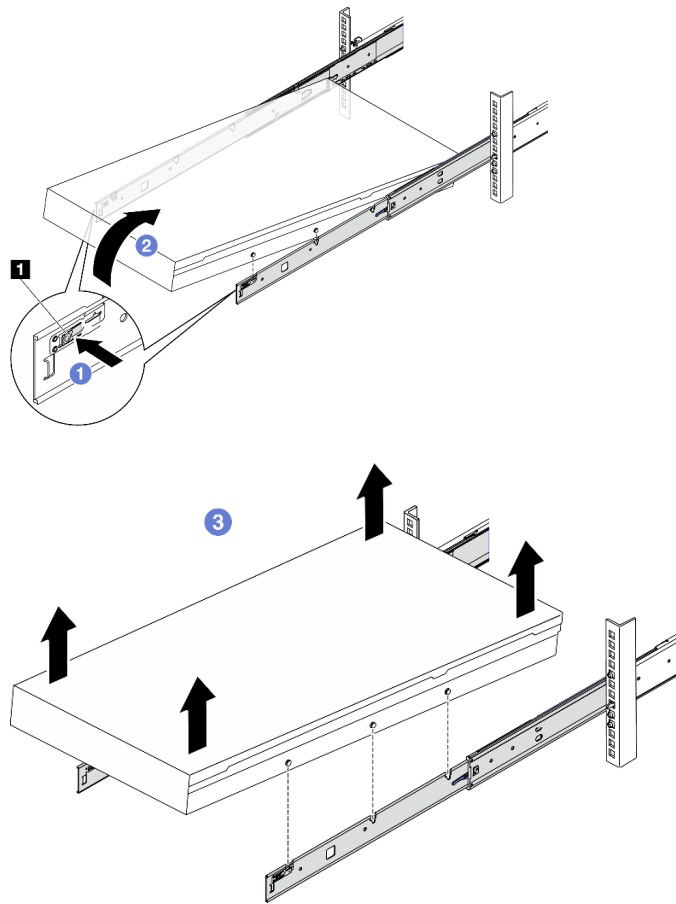
Figura 5. Extracción del servidor del bastidor
