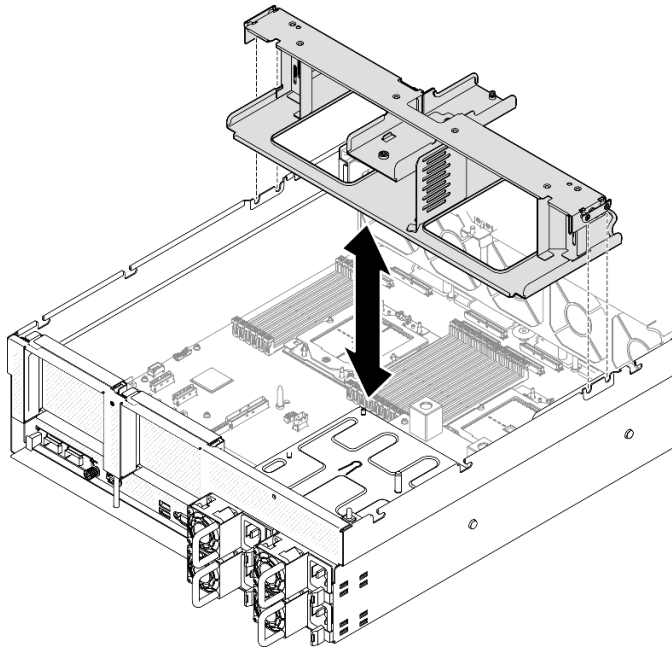
Figura 12. Extracción del deflector de aire
