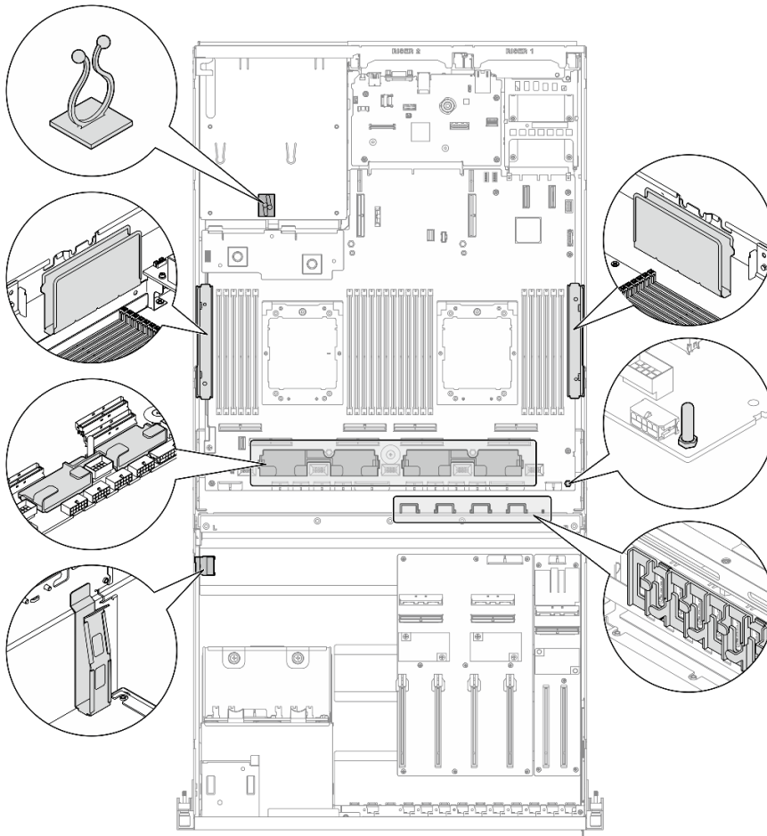
Figura 298. Ubicaciones de la guía de cables y del clip para cables en el chasis
