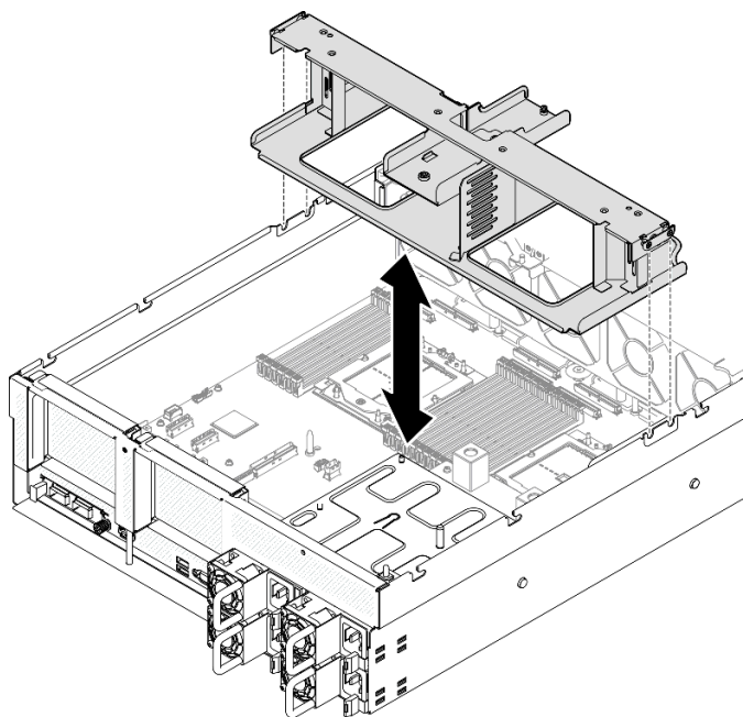
Figura 13. Instalación del deflector de aire
