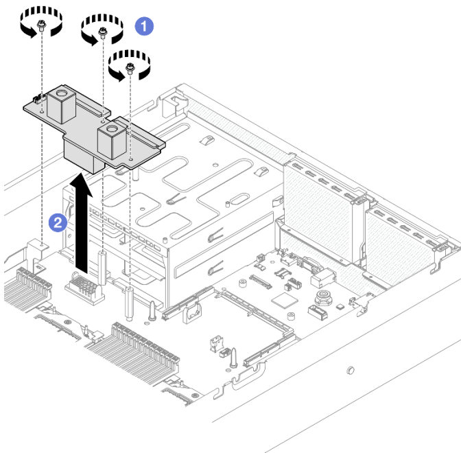
Figura 75. Extracción de la placa de distribución de alimentación
