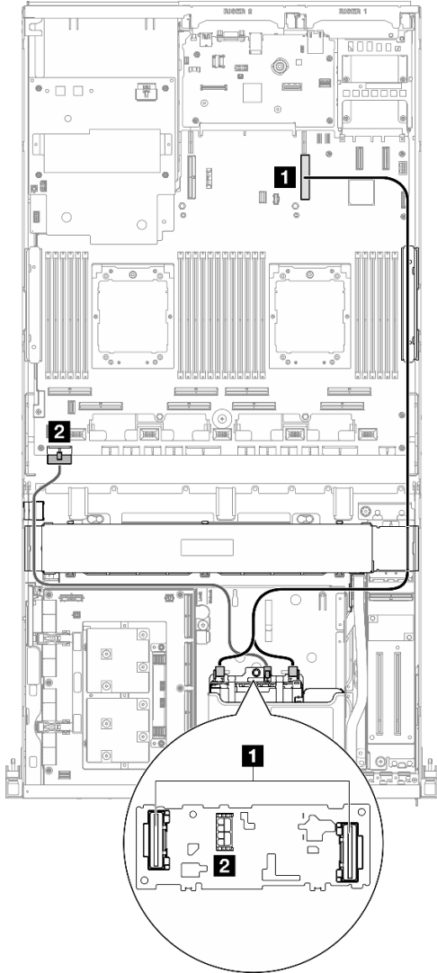
Figura 354. Disposición de los cables de la placa posterior de unidad E3.S
