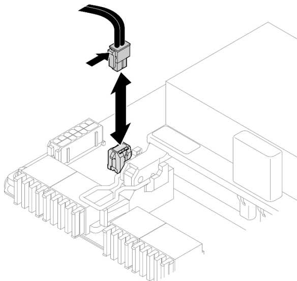
Figura 168. Desconexión del cable de alimentación
