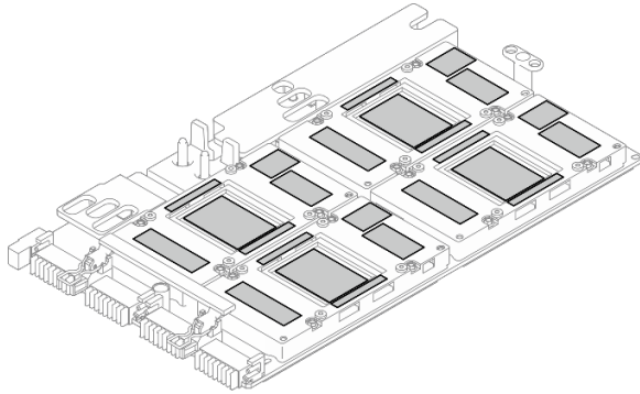
Figura 239. Limpieza del PCM y las almohadillas de masilla de las GPU SXM5
