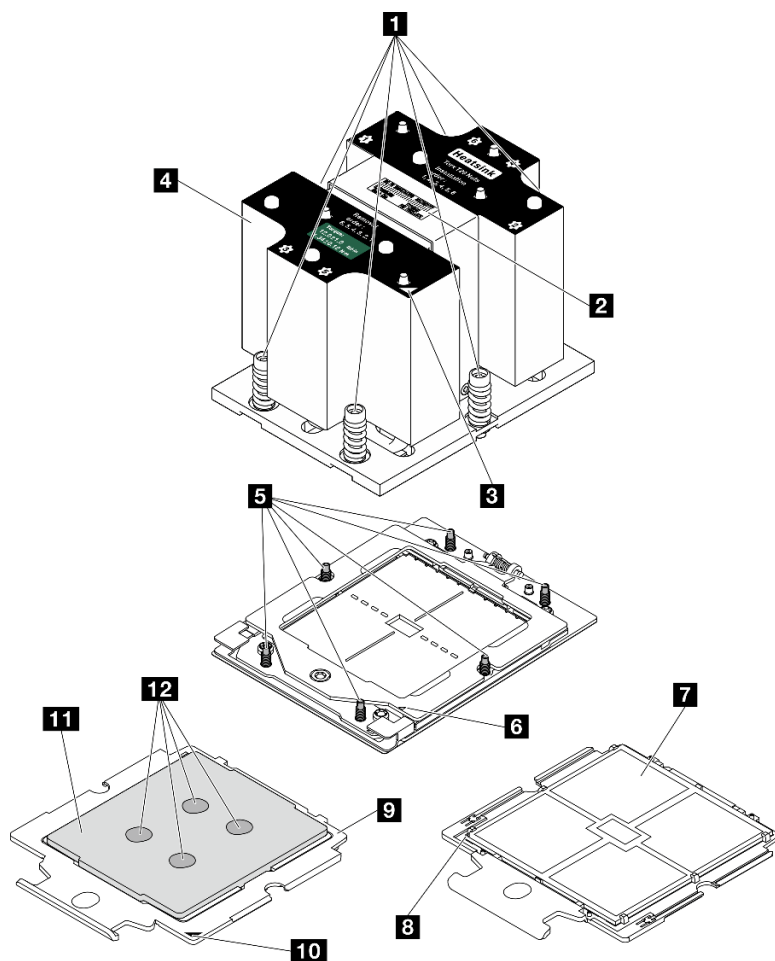
Figura 80. Componentes del procesador y el disipador de calor
