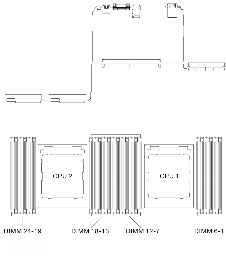
Figura 47. Diseño de los módulos de memoria y el procesador
