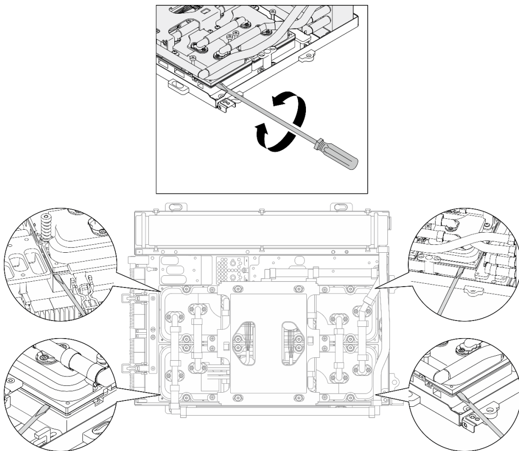
Figura 235. Desenganche de la placa de frío
