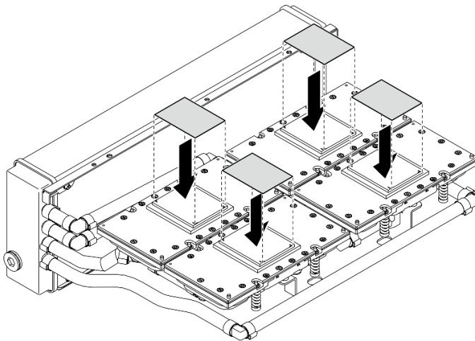
Figura 241. Aplicación de PCM
