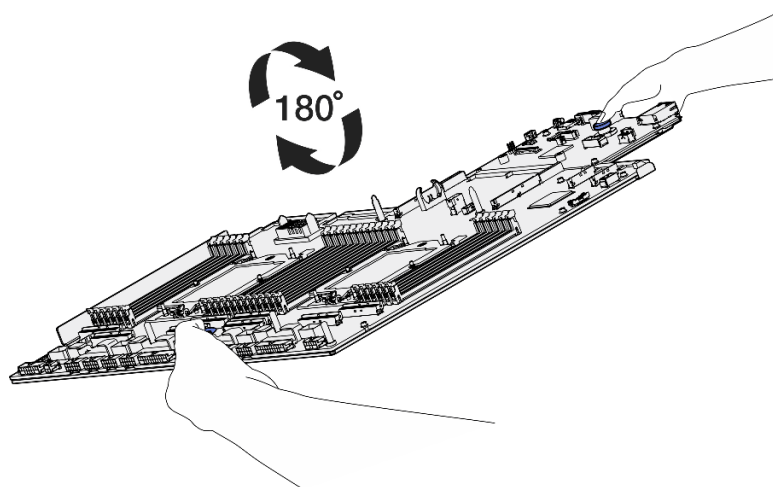
Figura 103. Giro del conjunto de la placa del sistema
