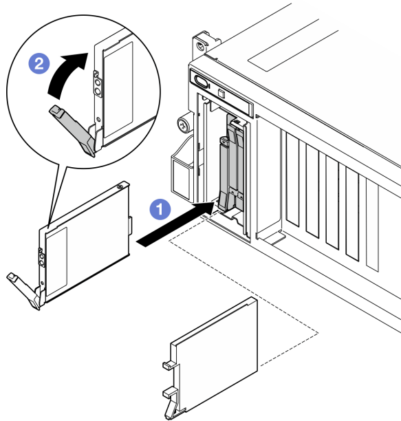
Figura 126. Instalación de una unidad de intercambio en caliente E3.S
