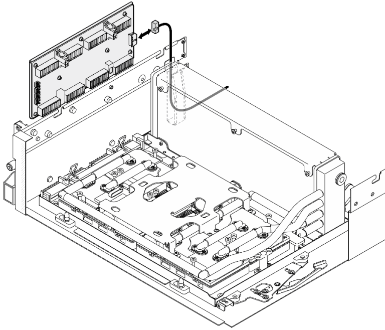
Figura 220. Desconexión del cable de alimentación de la tarjeta de interposición
