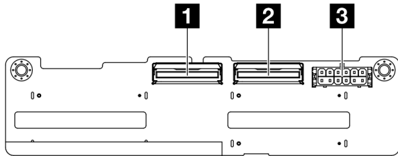
Figura 285. 4 conectores de placa posterior NVMe de 2,5 pulgadas
