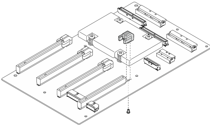
Figura 157. Instalación del refuerzo de una ranura de PCIe
