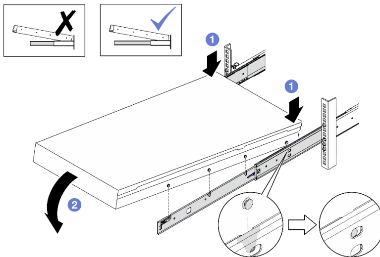
Figura 8. Instalación del servidor en los rieles
