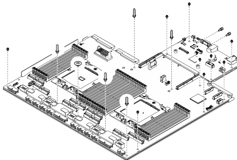
Figura 102. Instalación de componentes
