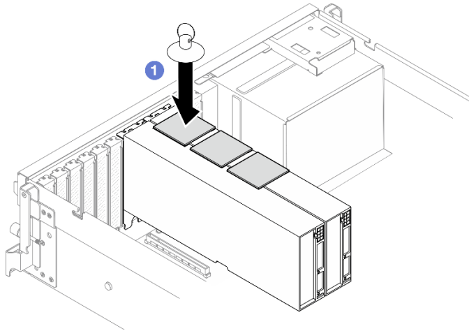
Figura 152. Extracción del Puente de enlace del adaptador de GPU
