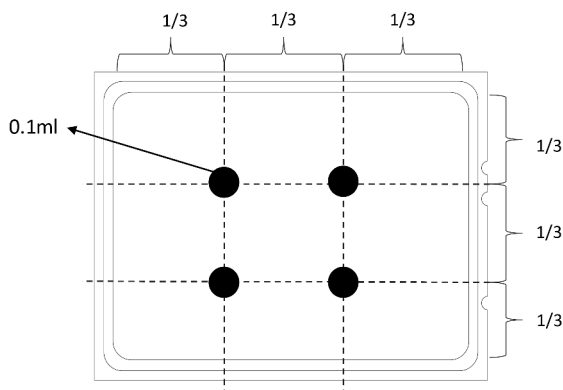
Figura 84. Aplicación de grasa térmica
