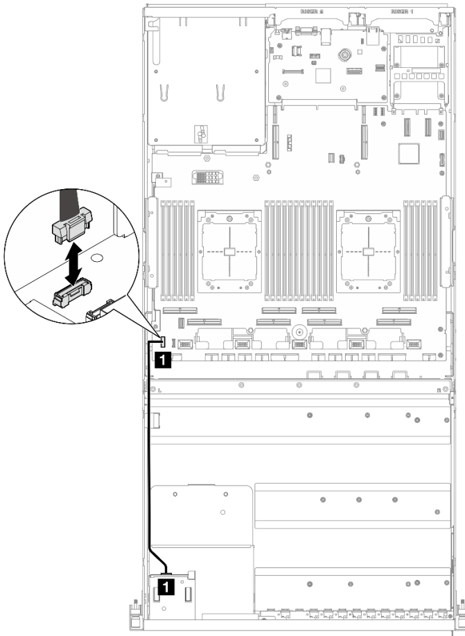
Figura 30. Desconexión del cable del panel frontal del operador - Modelo de GPU 4-DW y Modelo de GPU 8-DW
