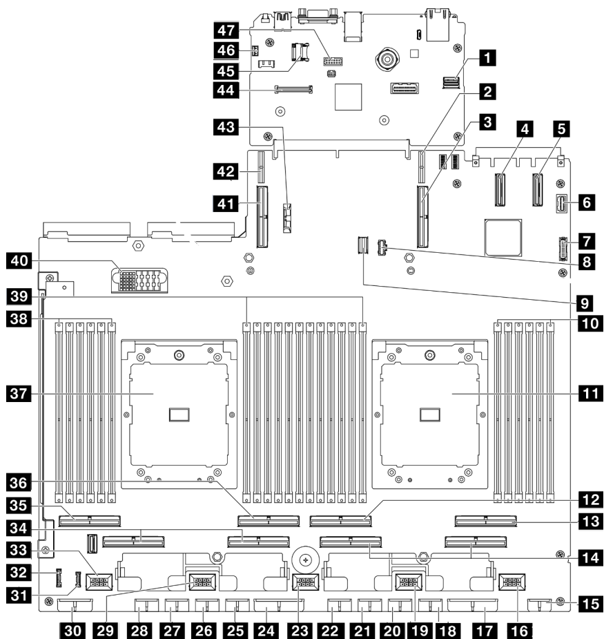
Figura 376. Conectores del conjunto de la placa del sistema
