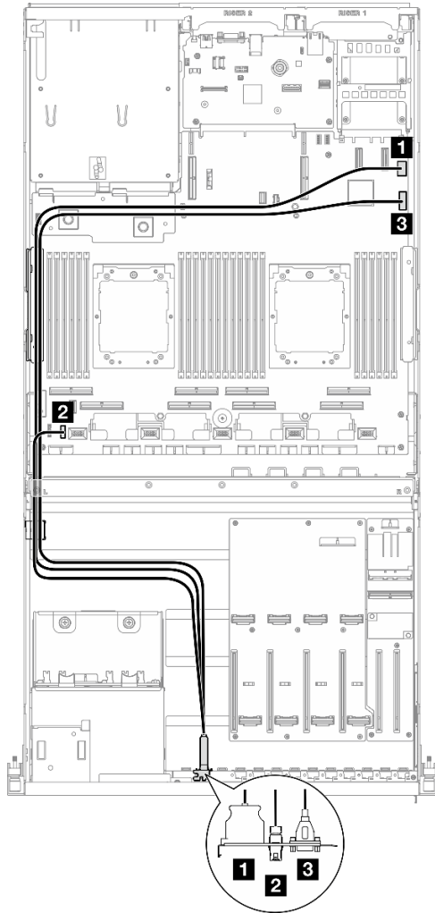
Figura 28. Disposición de los cables del módulo de E/S frontal - Modelo de GPU 4-DW
