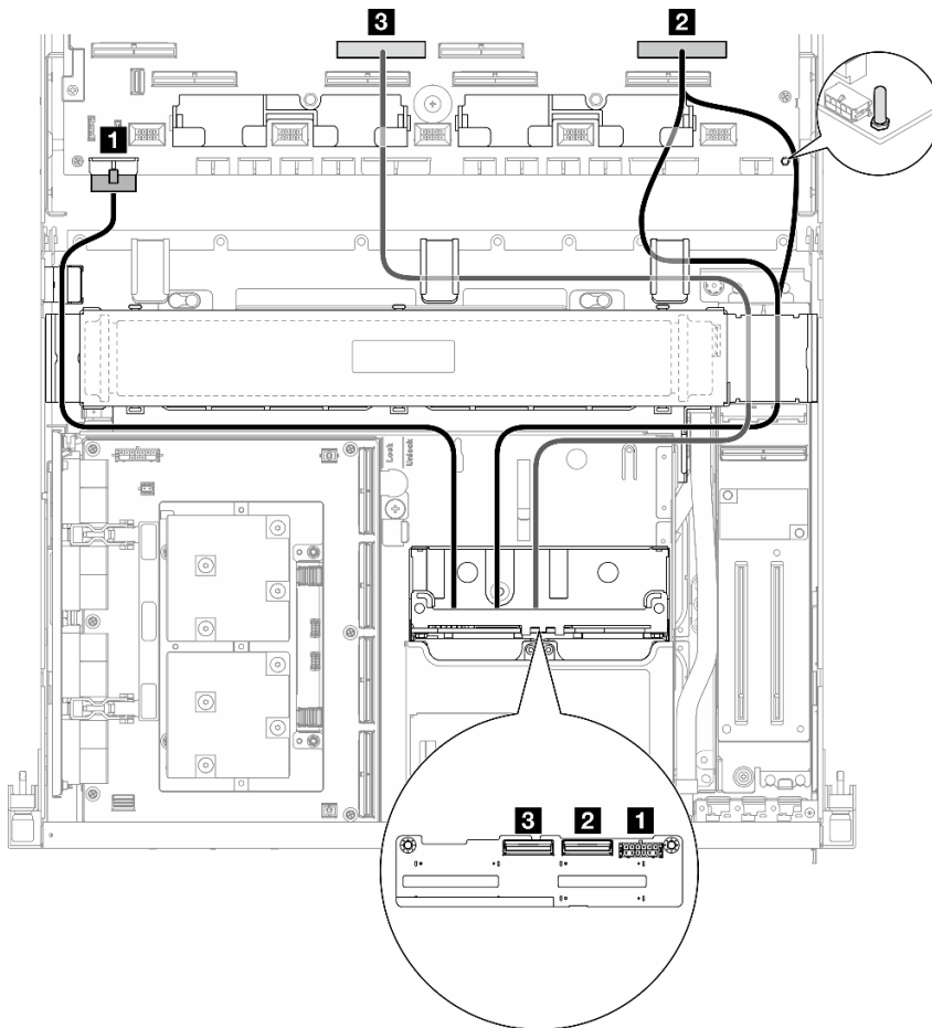
Figura 346. Disposición de los cables de la placa posterior de unidad de 2,5 pulgadas
