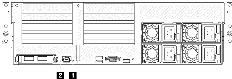
Figura 384. LED de sistema en la vista posterior
