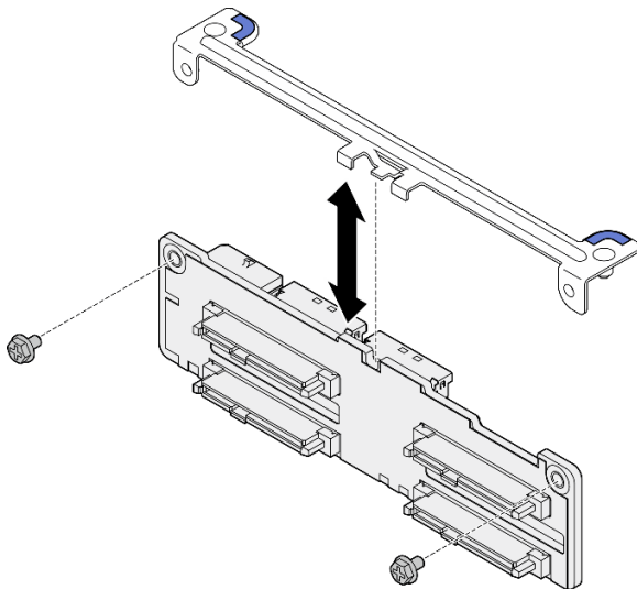
Figura 164. Extracción del soporte de la placa posterior de la unidad de 2,5 pulgadas
