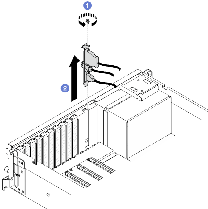
Figura 26. Extracción del módulo de E/S frontal
