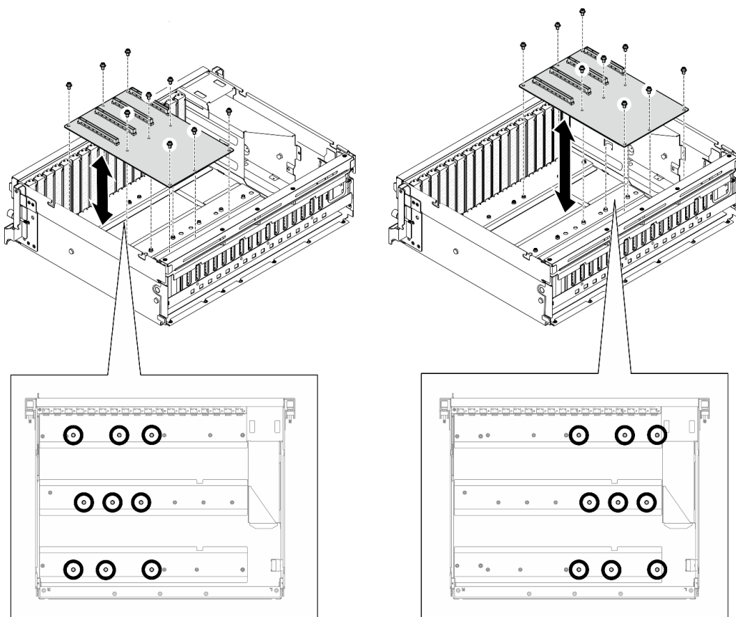
Figura 148. Extracción de la placa de distribución de GPU: Modelo de GPU 8-DW
