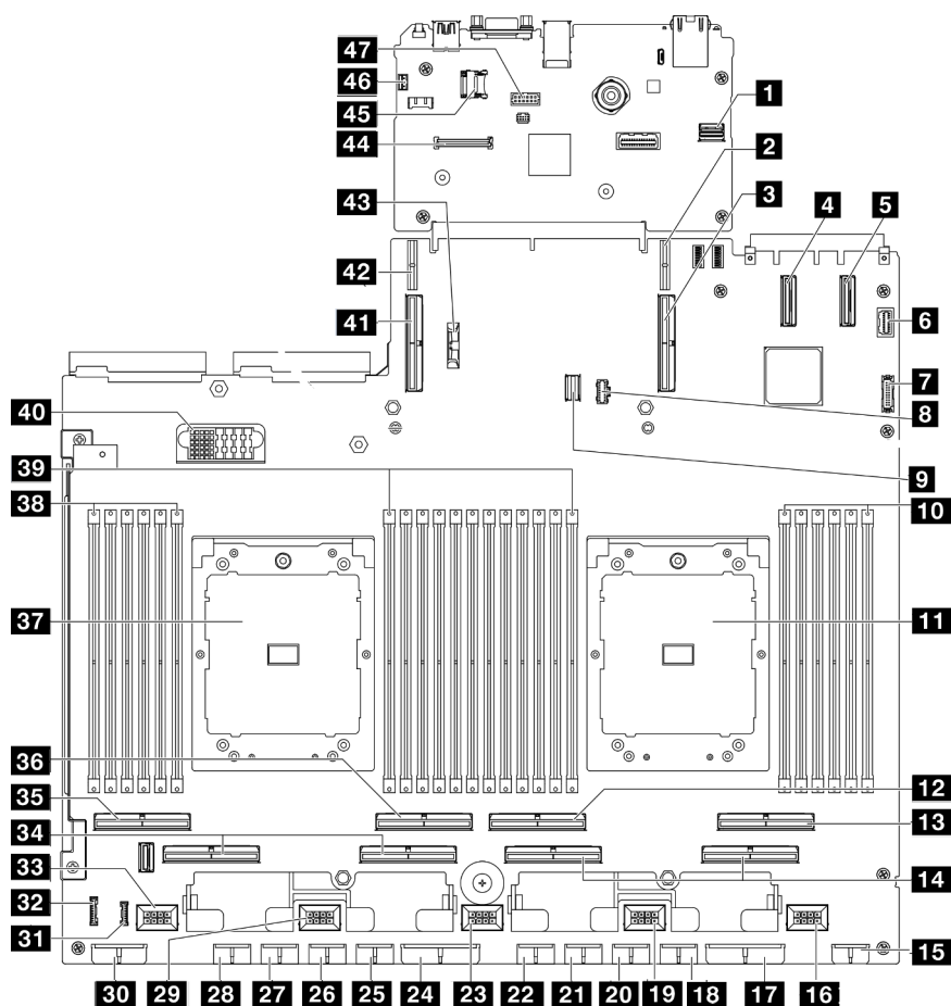
Figura 297. Conectores del conjunto de la placa del sistema
