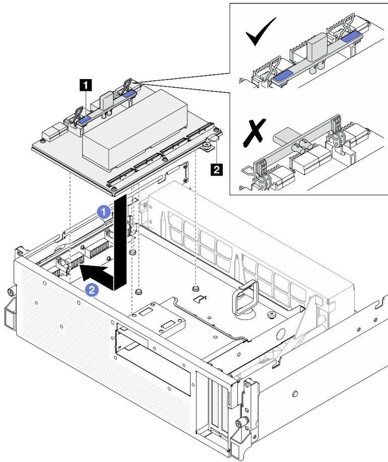
Figura 170. Instalación del Conjunto de CX-7
