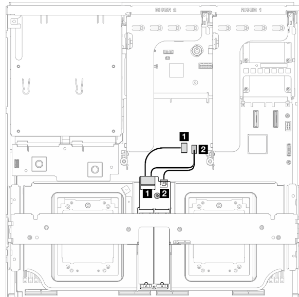
Figura 310. Disposición de cables para la placa posterior M.2 SATA/NVMe o RAID NVMe
