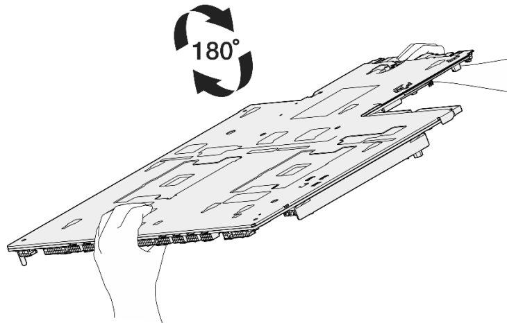
Figura 105. Giro del conjunto de la placa del sistema
