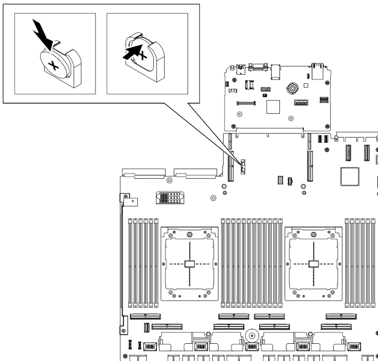
Figura 15. Instalación de la batería CMOS
