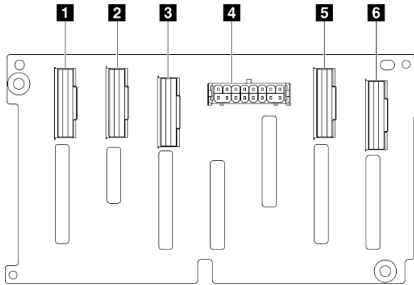
Figura 286. 8 conectores de placa posterior SAS/SATA/NVMe de 2,5 pulgadas
