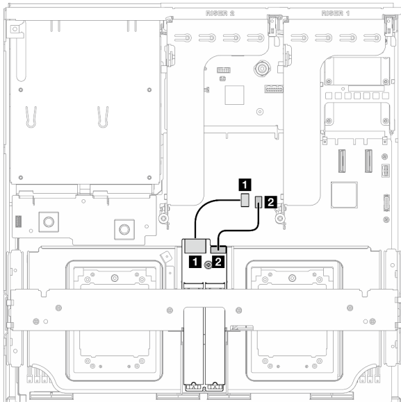
Figura 309. Disposición de los cables de la placa posterior M.2 SATA/x4 NVMe
