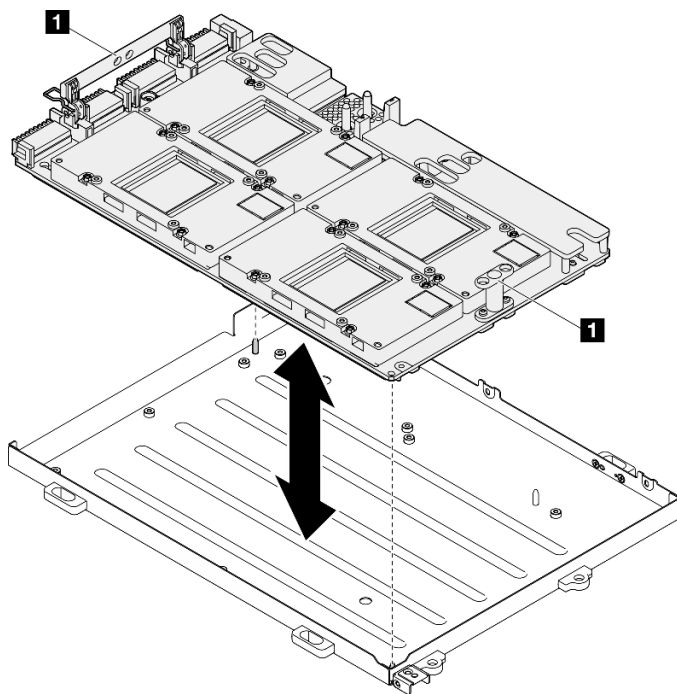
Figura 267. Instalación del Conjunto de placa de GPU SXM5
