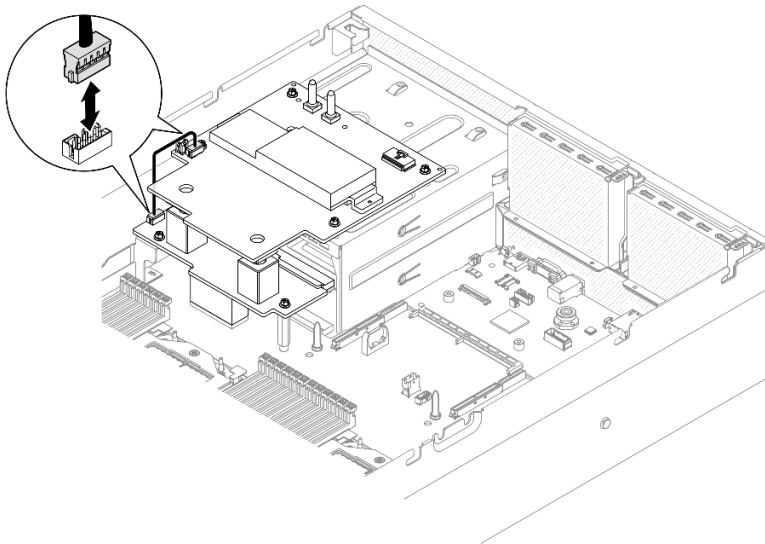
Figura 272. Desconexión del cable de banda lateral
