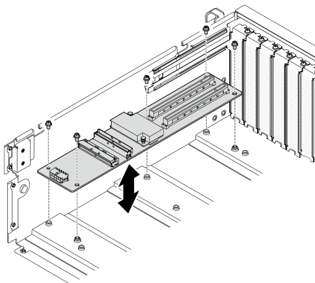
Figura 139. Extracción de la placa de expansión de E/S frontal
