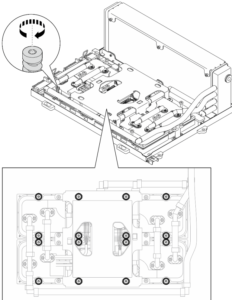
Figura 246. Instalación del tornillo Torx T15
