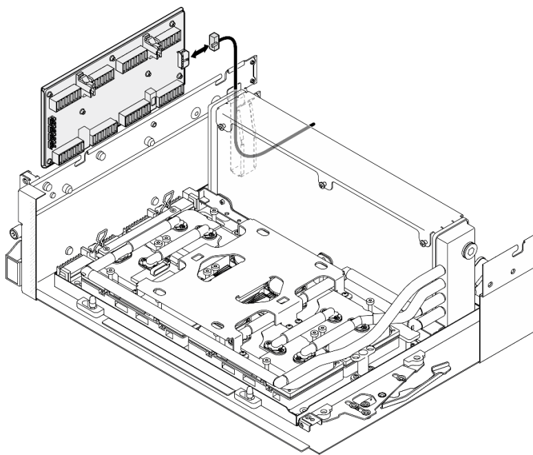
Figura 223. Conexión del cable de alimentación de la tarjeta de interposición
