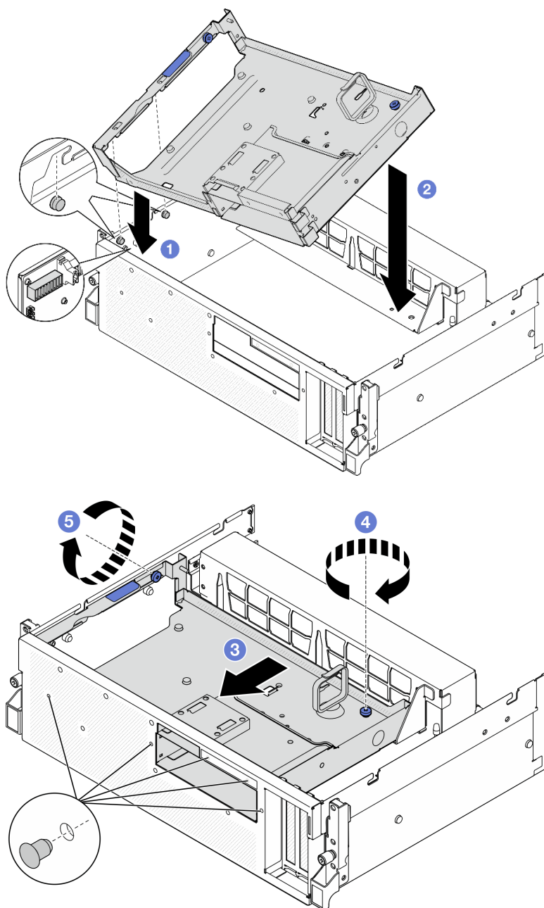
Figura 198. Instalación de la bandeja unidades frontal
