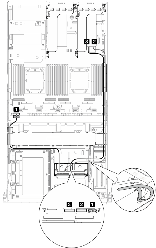
Figura 349. Disposición de los cables de la placa posterior de la unidad de 2,5 pulgadas (adaptador RAID en la expansión PCIe 1)
