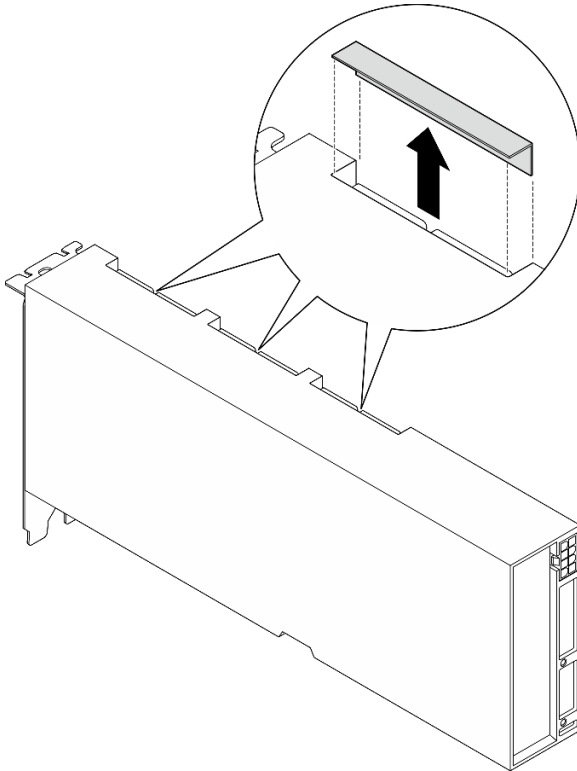
Figura 144. Extracción de la cubiertas del conector de enlace
