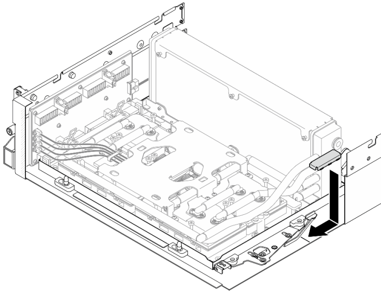
Figura 227. Instalación del soporte de sujeción del Conjunto de placa de GPU SXM5
