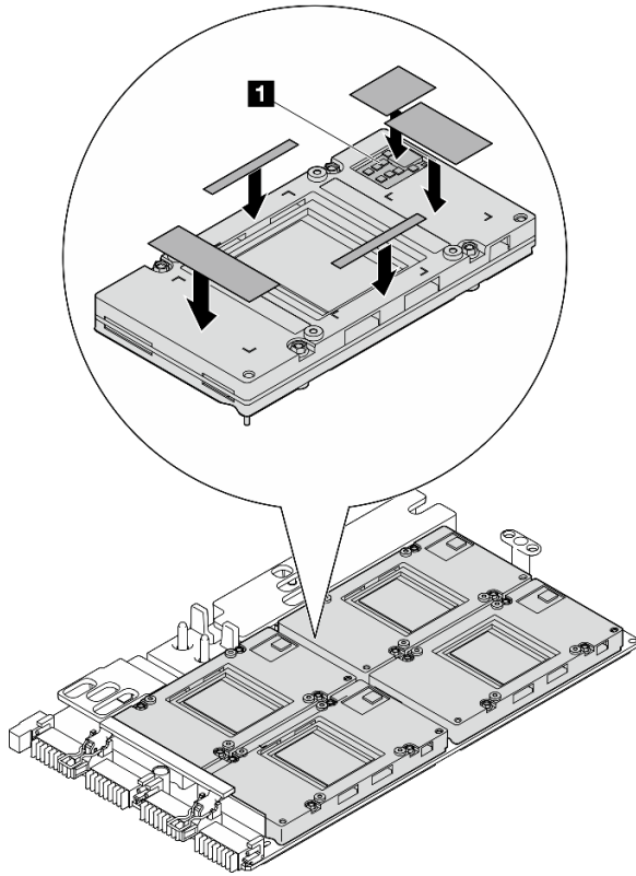
Figura 242. Aplicación de la almohadilla de masilla
