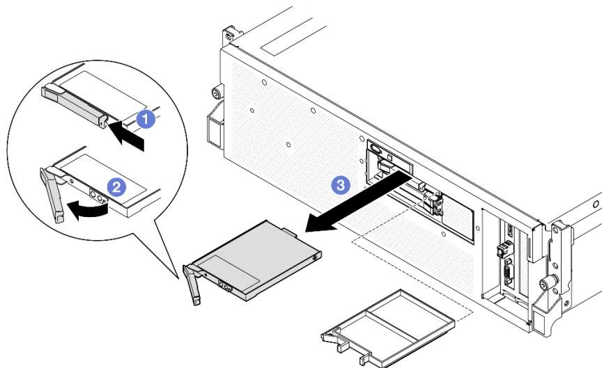
Figura 181. Extracción de una unidad de intercambio en caliente E3.S
