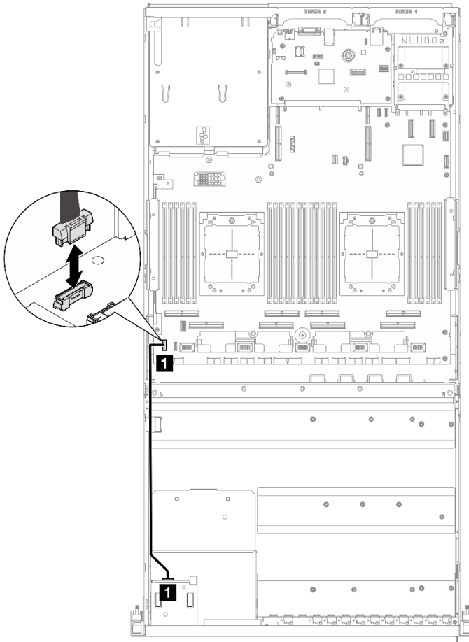
Figura 34. Disposición de los cables para el panel frontal del operador - Modelo de GPU 4-DW y Modelo de GPU 8-DW
