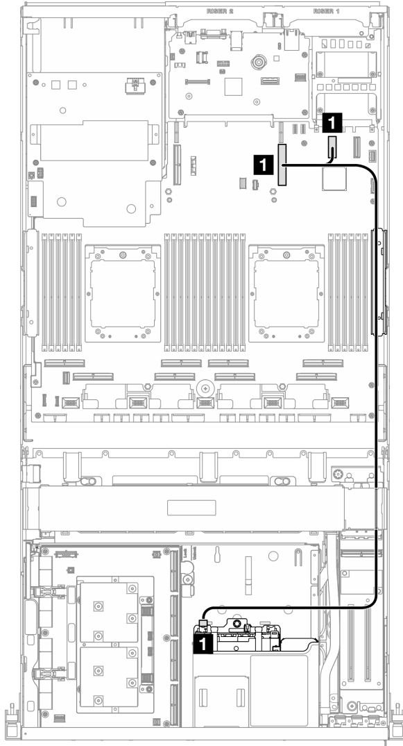
Figura 366. Disposición de los cables del módulo de OCP
