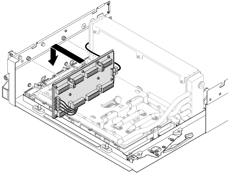
Figura 225. Instalación de la tarjeta de interposición
