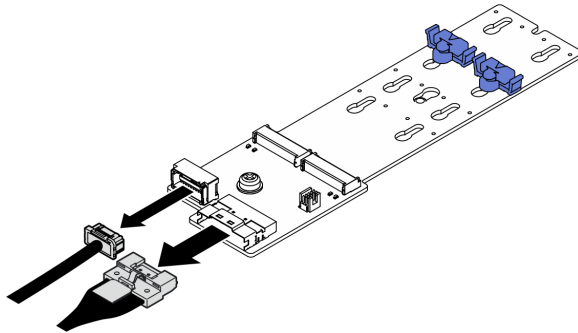
Figura 44. Conexión de cable de la placa posterior SATA/x4 NVMe M.2
