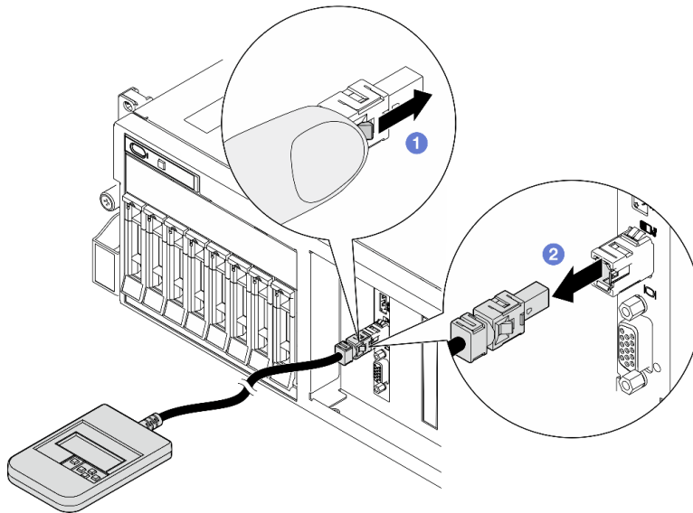
Figura 16. Desconexión del cable del auricular de diagnóstico externo
