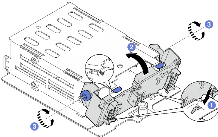
Figura 189. Instalación del módulo de la placa posterior de la unidad E3.S
