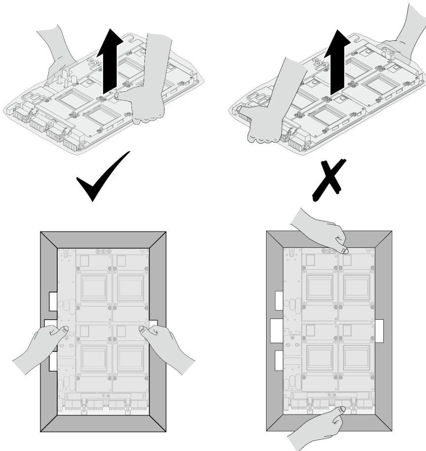
Figura 265. Extracción de la Conjunto de placa de GPU SXM5 de la caja del paquete
