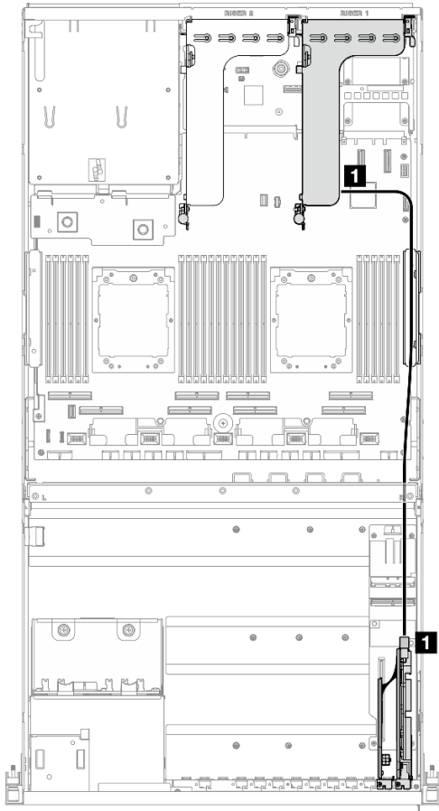
Figura 303. Disposición de los cables de alimentación del Adaptador DPU
