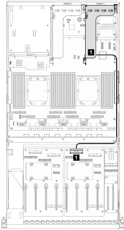
Figura 333. Disposición de los cables de la expansión de PCIe 1
