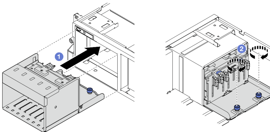
Figura 117. Instalación de un conjunto de compartimiento de una unidad de 2,5 pulgadas
