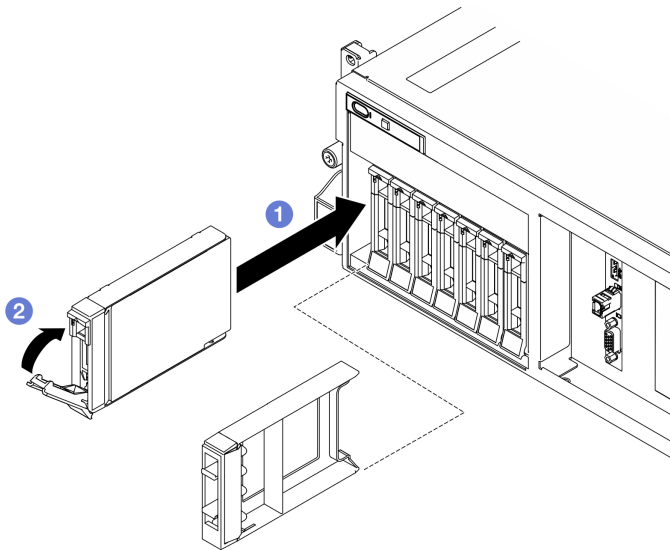
Figura 113. Instalación de unidad de intercambio en caliente de 2,5 pulgadas
