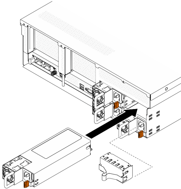
Figura 79. Instalación de la unidad de fuente de alimentación
