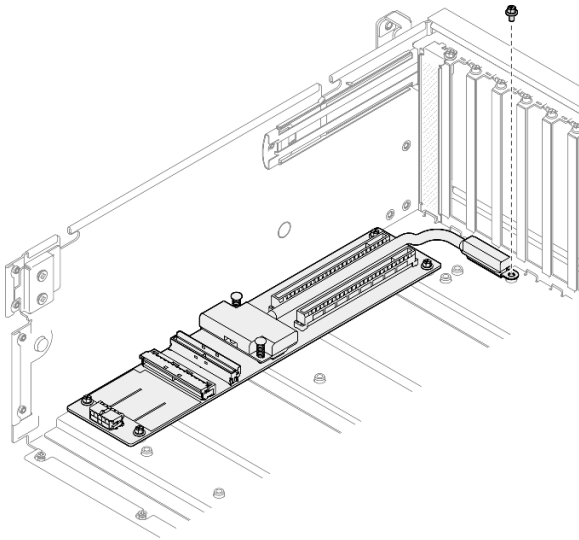
Figura 141. Instalación del tornillo
