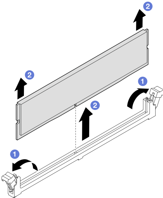
Figura 49. Extracción del módulo de memoria
