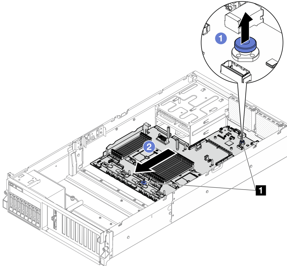
Figura 91. Desenganche del conjunto de la placa del sistema
