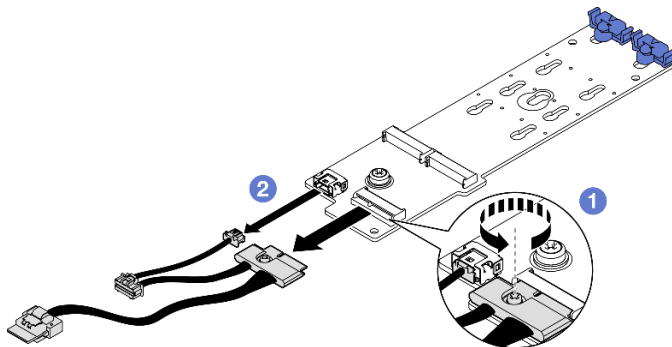
Figura 41. Desconexión del cable de la placa posterior M.2 SATA/NVMe o RAID NVMe
