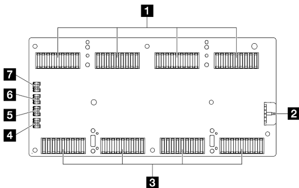
Figura 292. Conectores de la tarjeta de interposición
