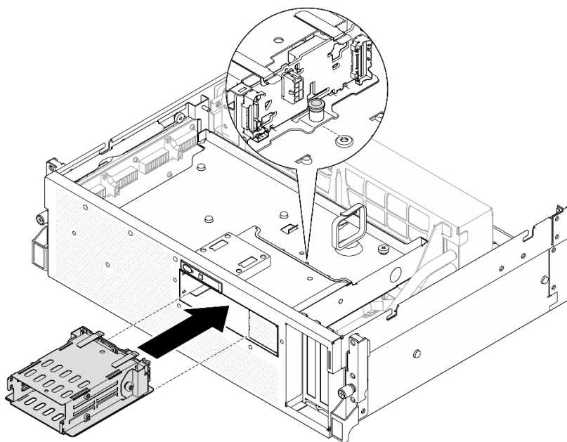
Figura 191. Instalación de un conjunto de compartimiento de una unidad E3.S
