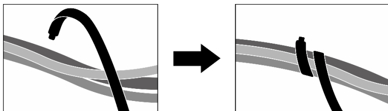
Figura 352. Fijación de los cables con las bridas de cables
