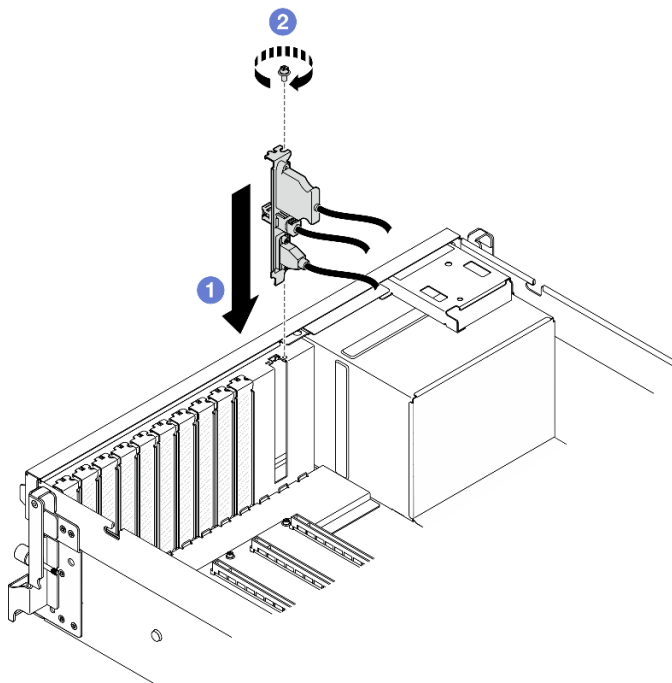
Figura 27. Instalación del módulo de E/S frontal
