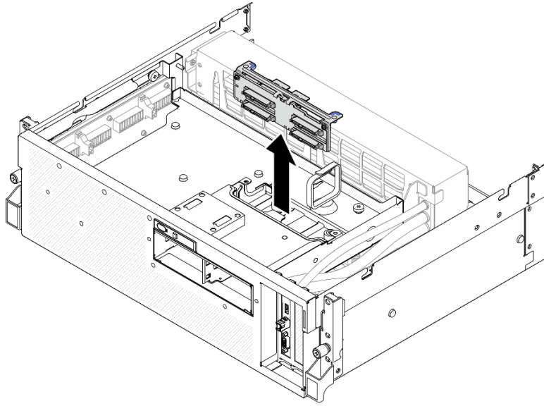
Figura 163. Extracción del módulo de la placa posterior de la unidad de 2,5 pulgadas
