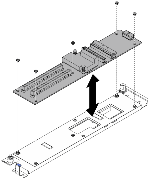
Figura 204. Instalación de la placa de expansión de E/S frontal
