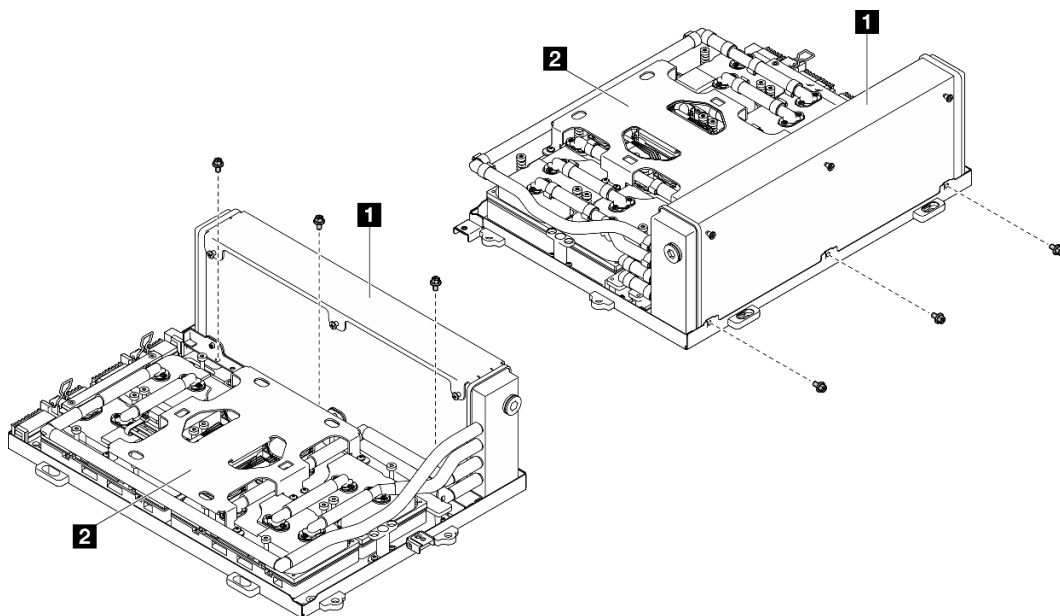
Figura 233. Extracción del tornillo Phillips n.º 1
