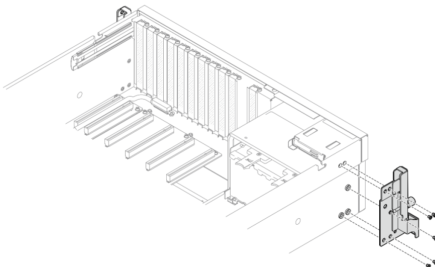
Figura 58. Instalación del tornillo de montaje izquierdo
