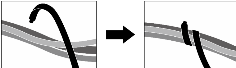
Figura 270. Fijación de los cables con las bridas de cables
