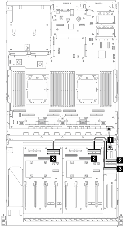
Figura 323. Disposición de los cables de la placa de expansión de E/S frontal
