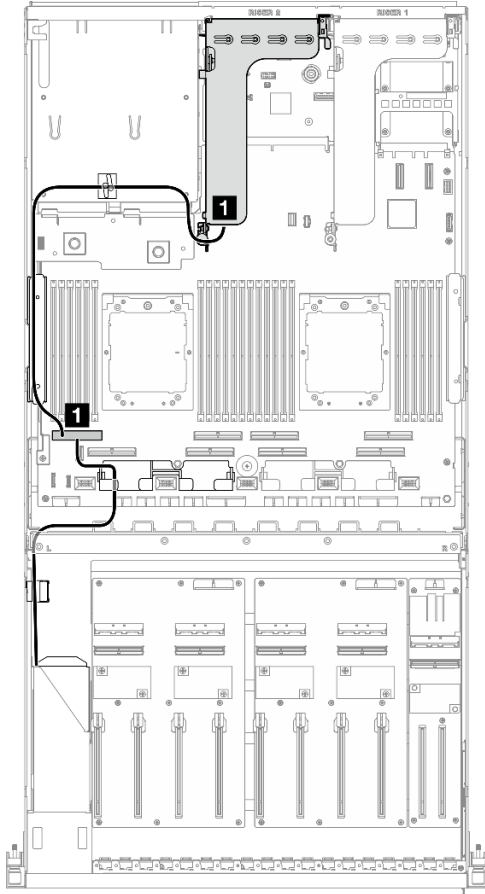
Figura 335. Disposición de los cables de la expansión de PCIe 2
