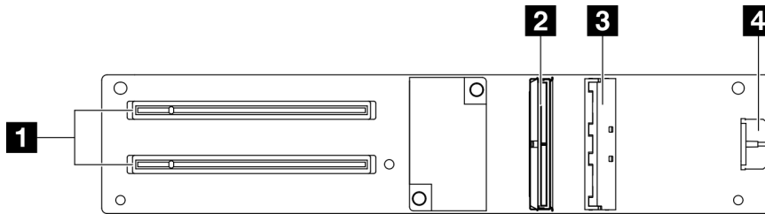
Figura 291. Conectores de la placa de expansión de E/S frontal
