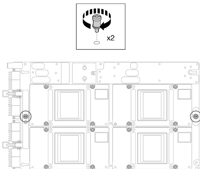
Figura 269. Instalación del tornillo T15
