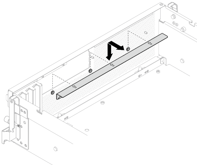
圖例 215. 卸下前方磁碟機托盤支撐托架
