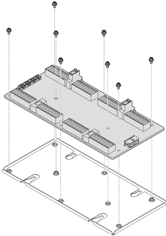
圖例 221. 拆卸轉插卡
