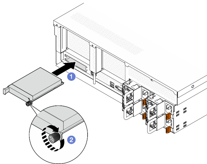
圖例 60. OCP 模組安裝
