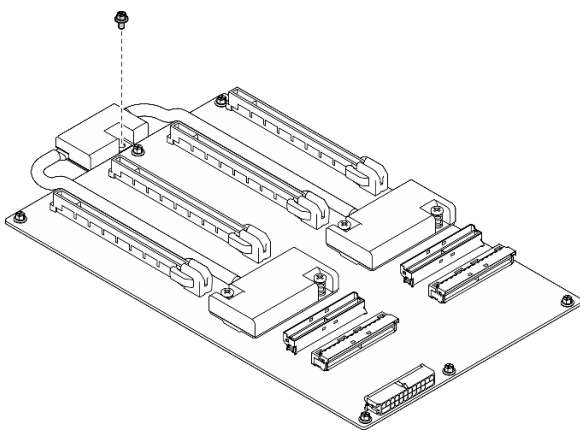
圖例 151. 安裝螺絲
