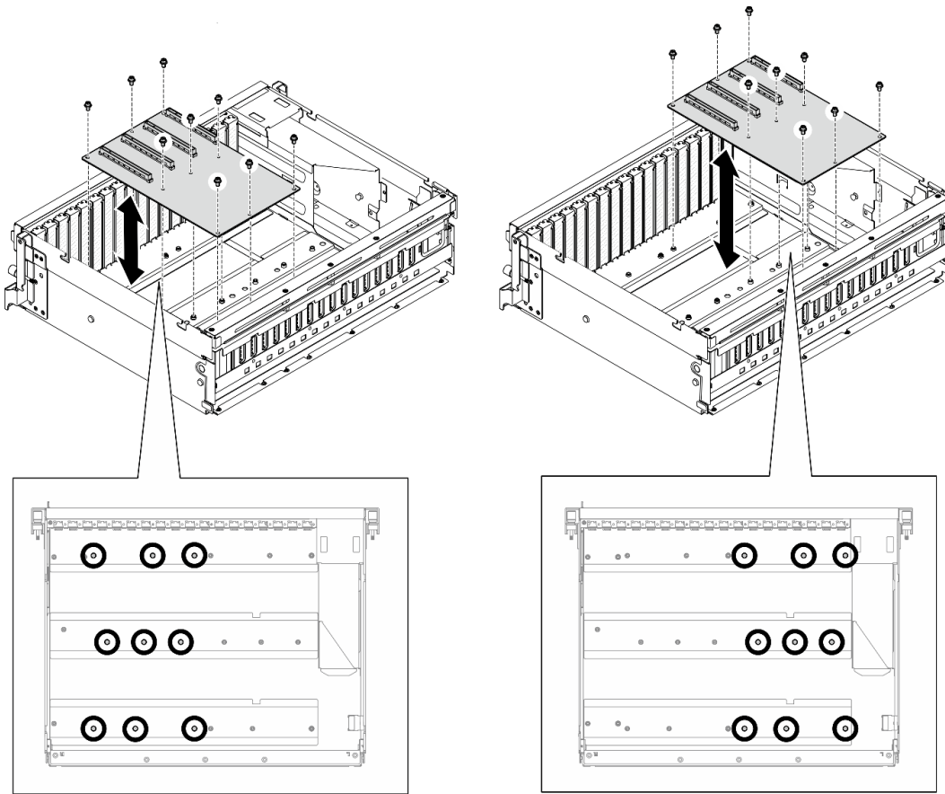
圖例 150. 安裝 GPU 配電板 — 8-DW GPU 型號
