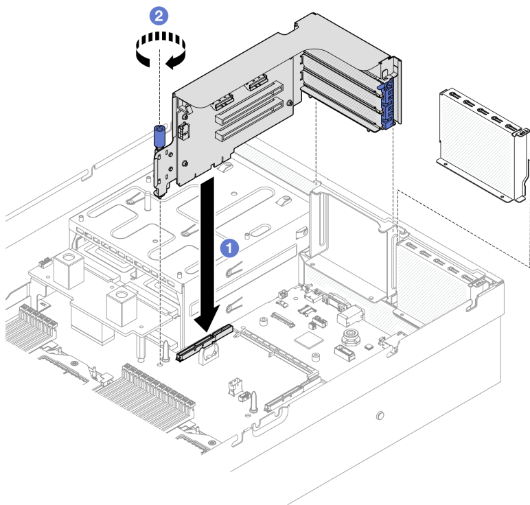
圖例 70. 安裝 PCIe 擴充卡 (不含序列埠模組)
