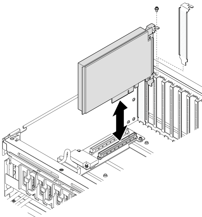
圖例 63. 安裝正面 PCIe 配接卡
