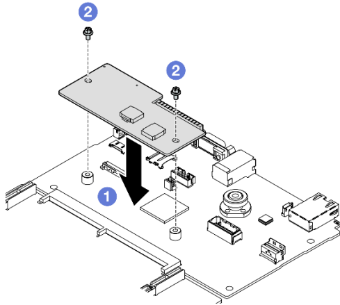
圖例 90. 安裝韌體和 RoT 安全模組
