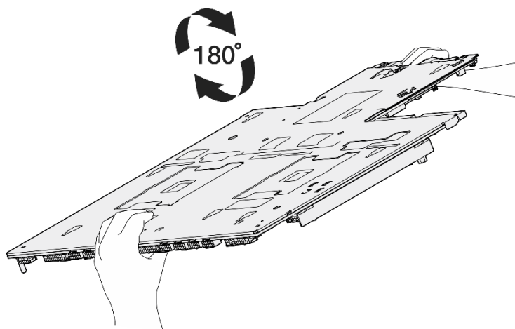
圖例 96. 翻轉主機板組件
