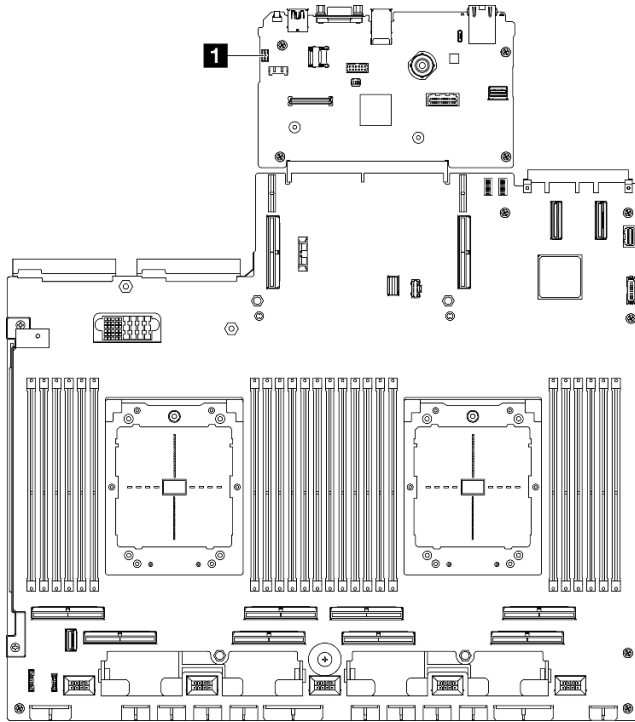
圖例 38. 入侵開關接頭位置
