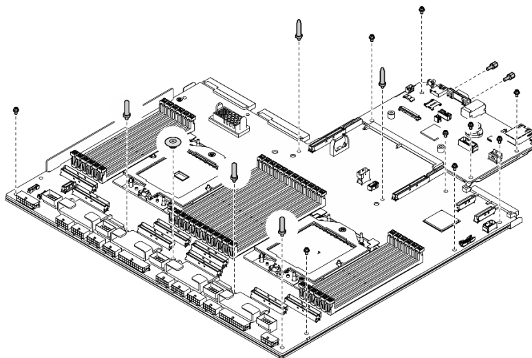
圖例 97. 卸下元件
