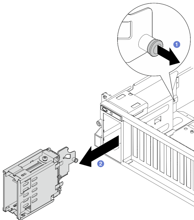
圖例 135. 卸下 E3.S 框架組件
