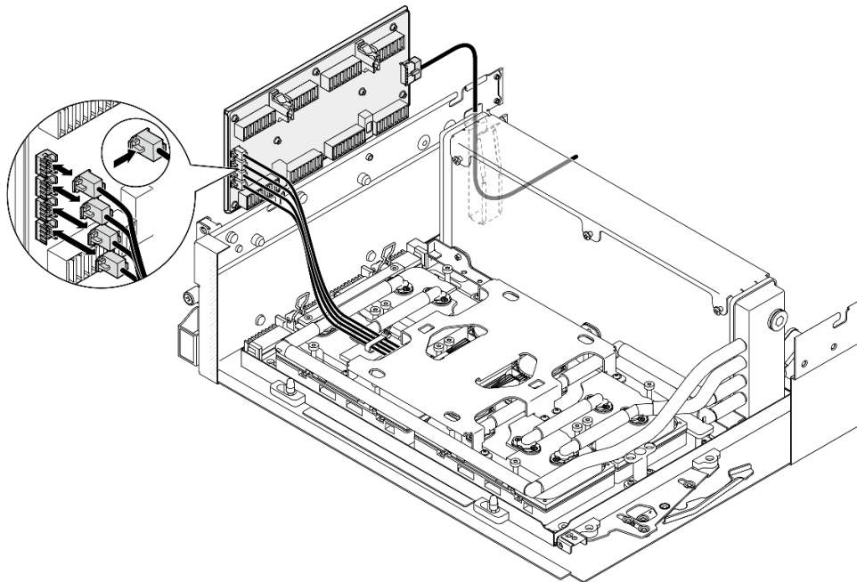
圖例 219. 拔除水冷板組件幫浦纜線
