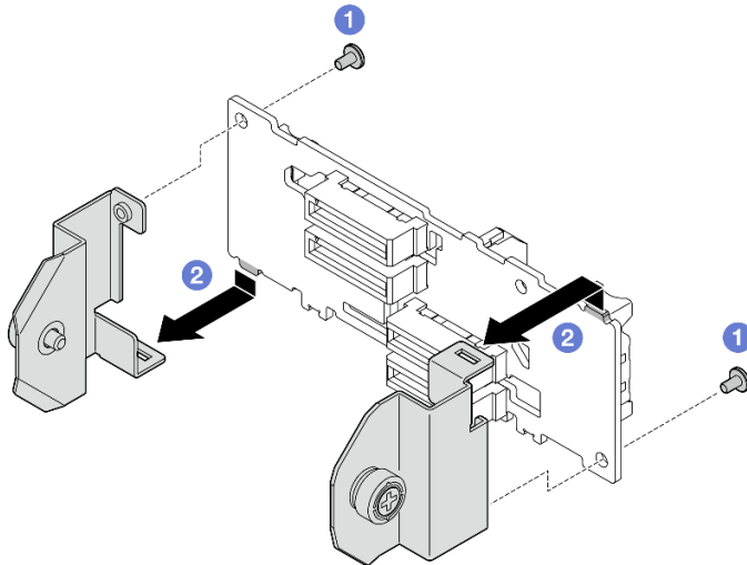
圖例 187. 卸下 E3.S 硬碟背板托架
