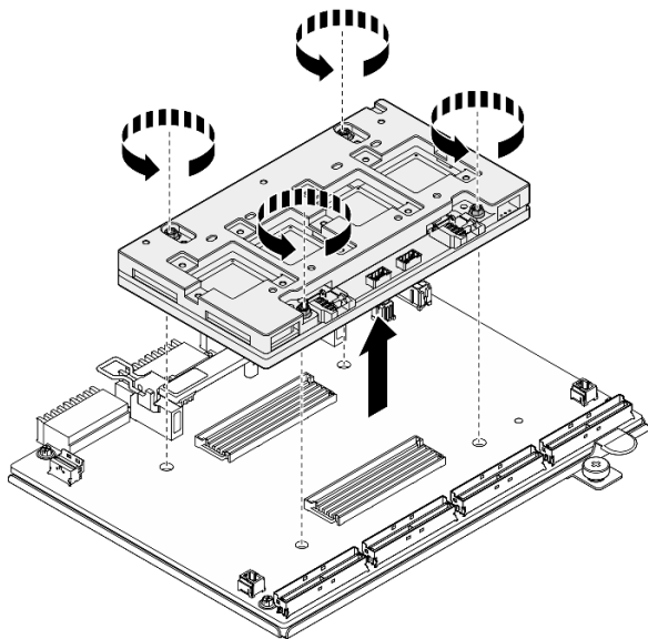
圖例 172. 卸下CX-7 Mezz 板
