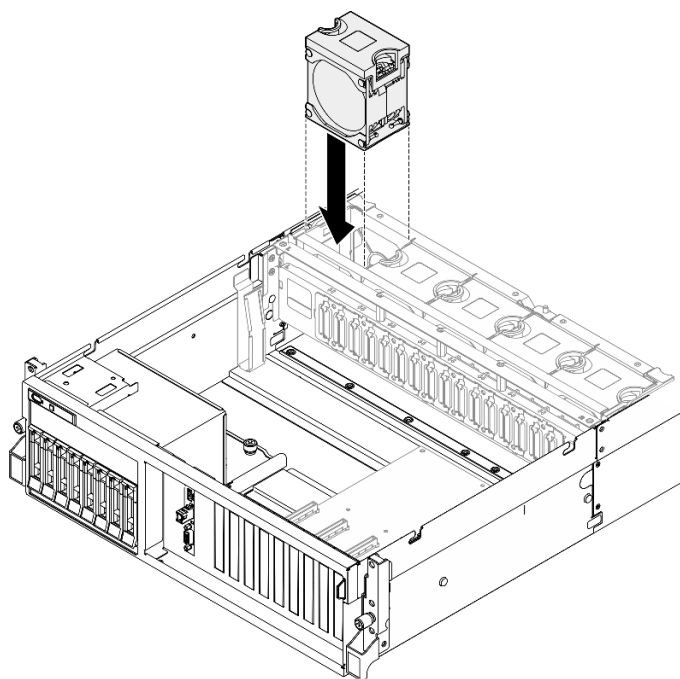
圖例 20. 安裝風扇
