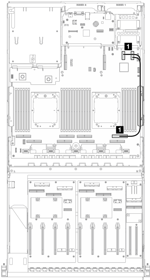
圖例 331. OCP 模組纜線佈線
