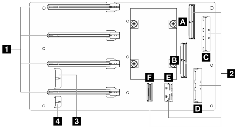
圖例 290. 已切換的 GPU 配電板 接頭
