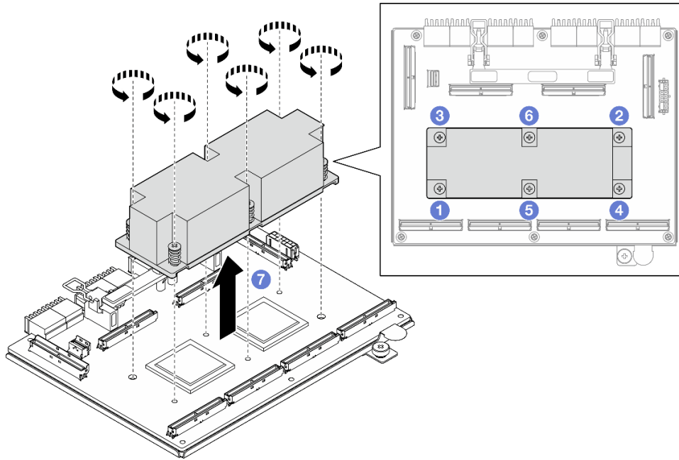
圖例 280. 卸下 SXM5 PCIe 交換器板散熱槽
