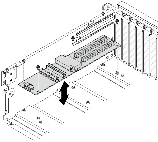
圖例 140. 安裝正面 I/O 擴充板
