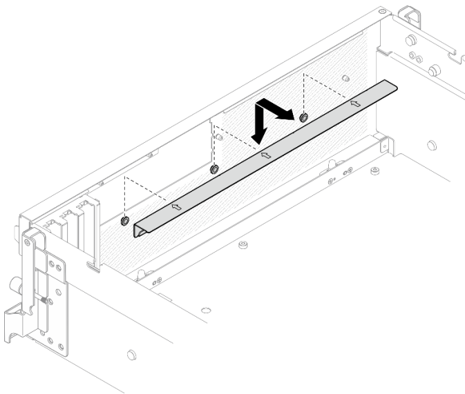
圖例 228. 安裝前方磁碟機托盤支撐托架
