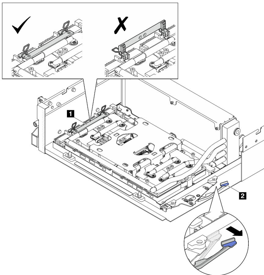
圖例 222. GPU-L2A 組件調整
