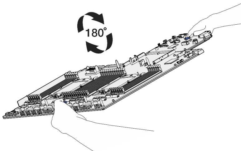
圖例 103. 翻轉主機板組件
