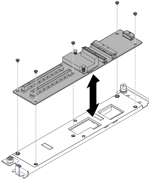
圖例 203. 卸下正面 I/O 擴充板
