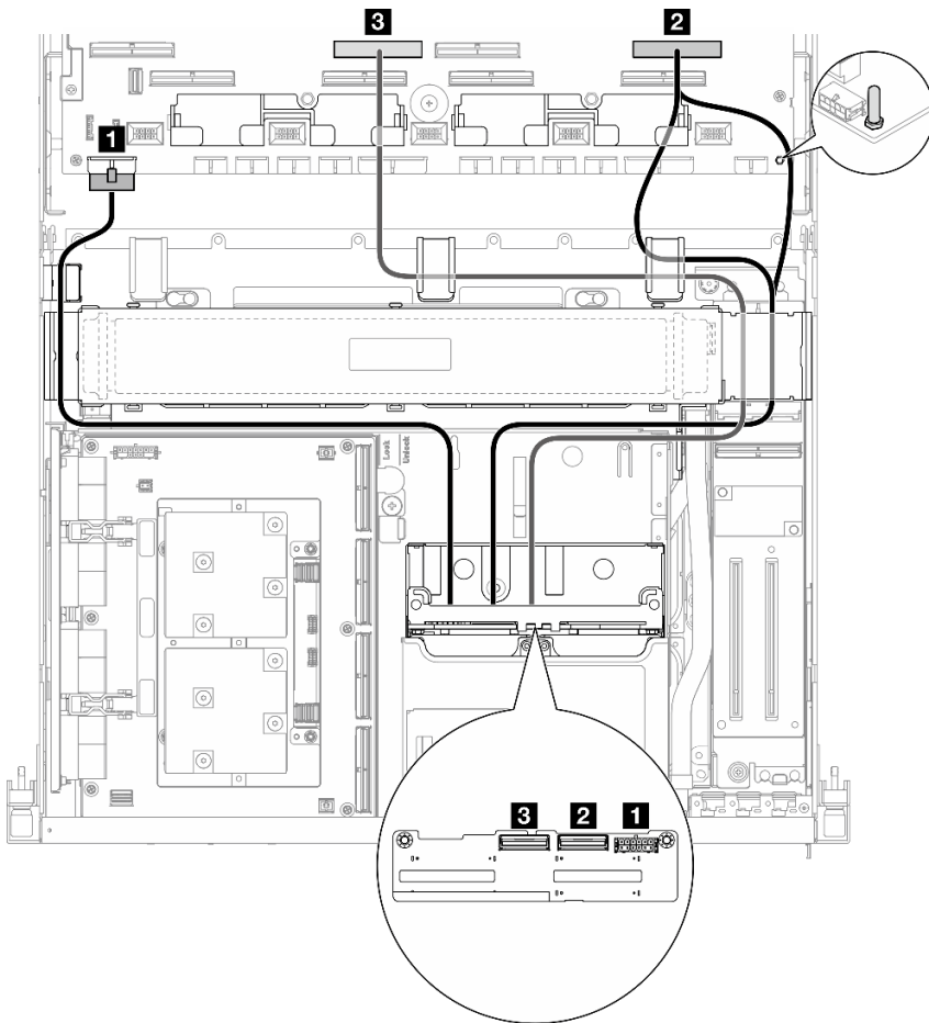
圖例 346. 2.5 吋硬碟背板纜線佈線
