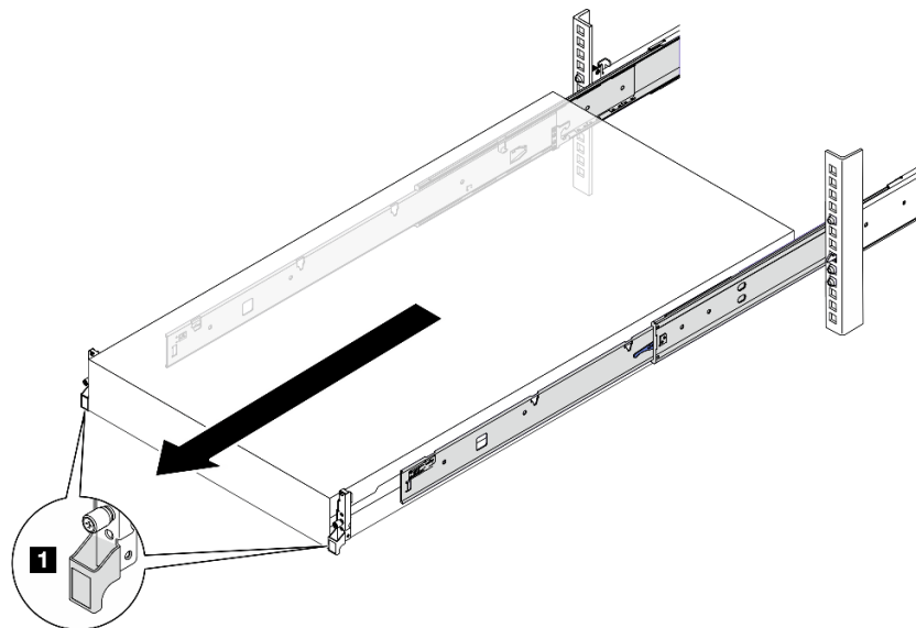
圖例 3. 拉出伺服器
