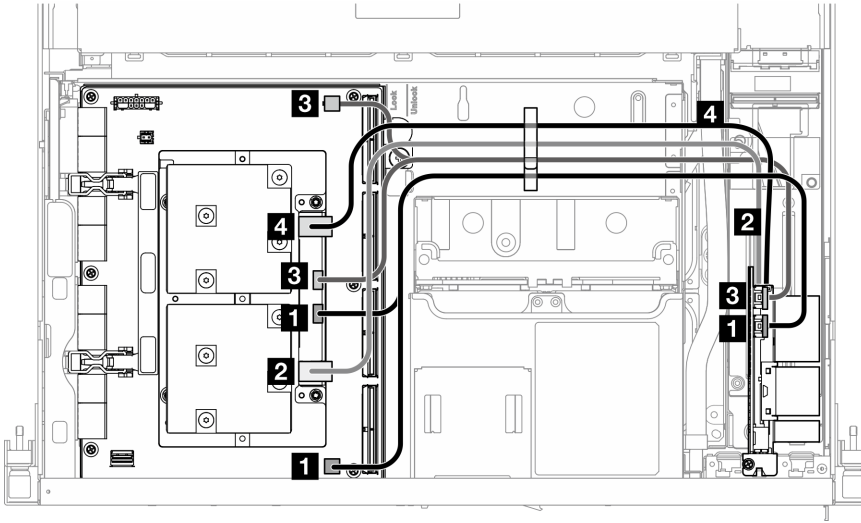
圖例 370. OSFP 埠卡纜線佈線
