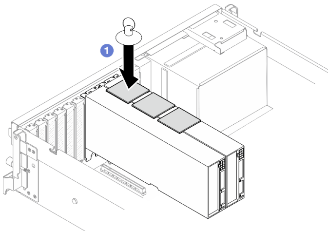
圖例 152. 卸下 GPU 配接卡鏈結橋接器
