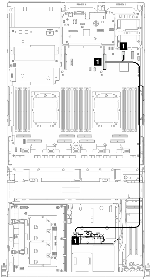
圖例 366. OCP 模組纜線佈線
