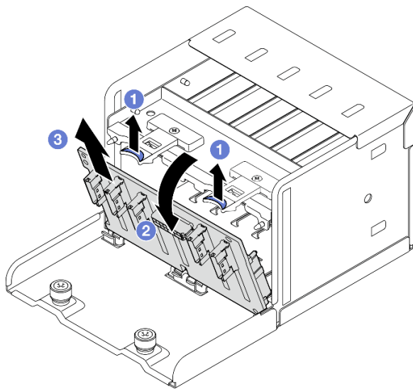
圖例 114. 卸下 2.5 吋硬碟背板
