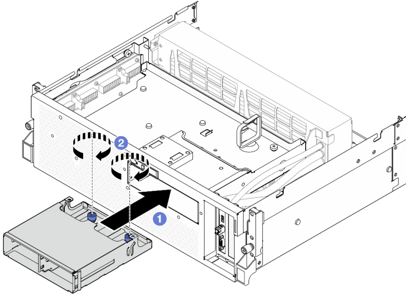
圖例 167. 安裝 2.5 吋框架
