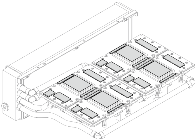
圖例 238. 擦掉水冷板上的 PCM 和油灰墊
