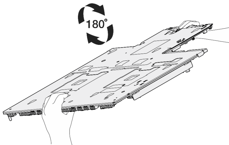
圖例 105. 翻轉主機板組件
