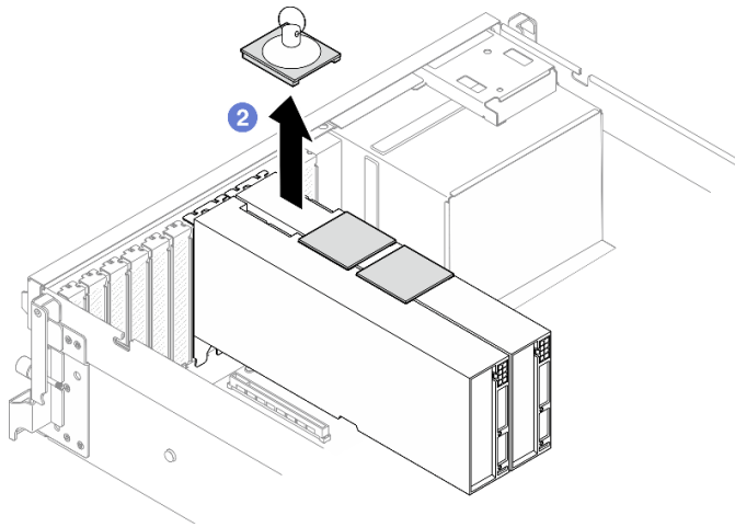
圖例 153. 卸下GPU 配接卡鏈結橋接器
