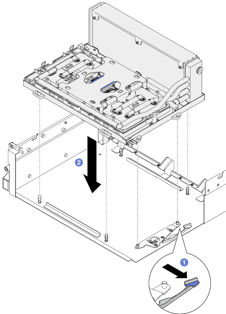
圖例 247. 安裝 GPU-L2A 組件
