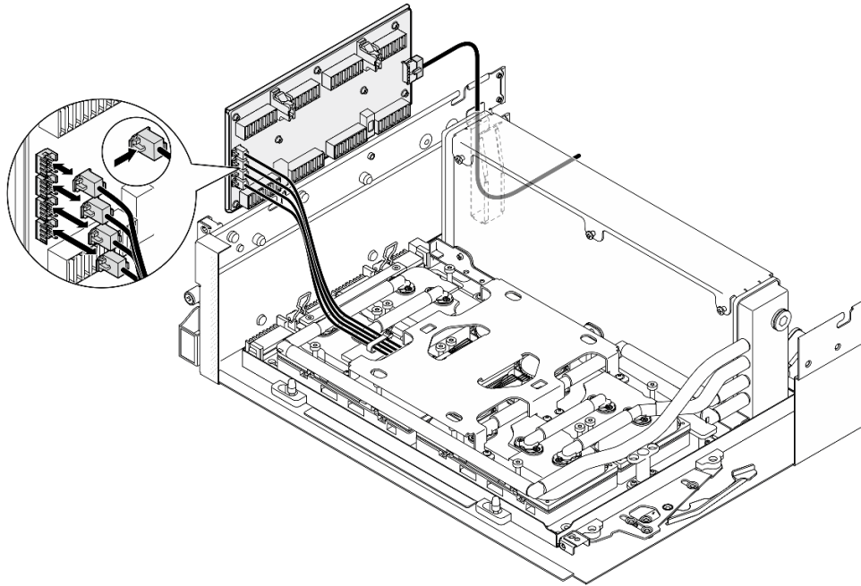
圖例 224. 水冷板組件幫浦纜線連接
