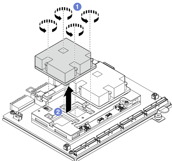
圖例 176. 卸下 CX-7 散熱槽
