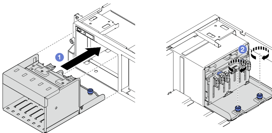
圖例 117. 安裝 2.5 吋框架組件
