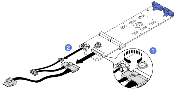
圖例 41. 拔除 SATA/NVMe 或 NVMe RAID M.2 背板纜線
