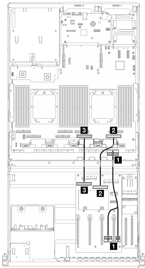
圖例 308. 已切換的 GPU 配電板纜線佈線
