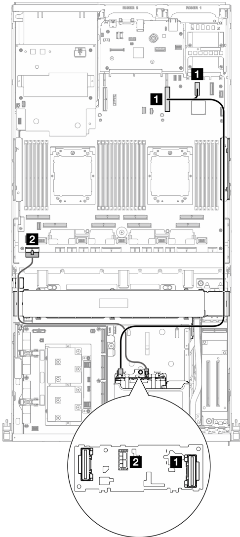
圖例 353. E3.S 硬碟背板纜線佈線
