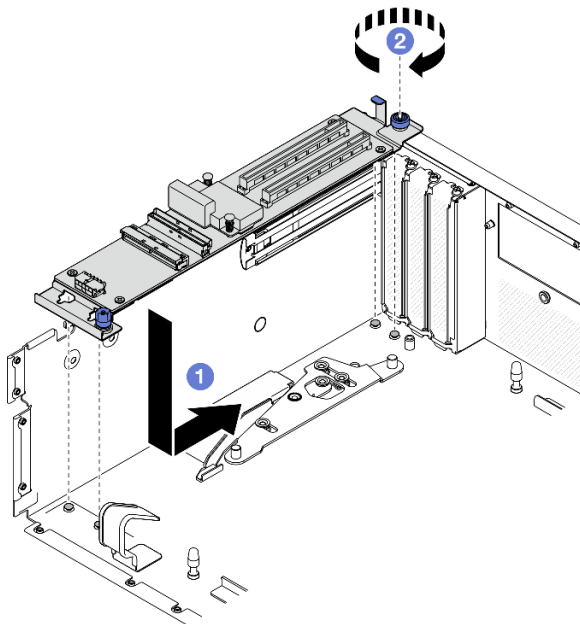
圖例 205. 安裝正面 I/O 擴充板模組
