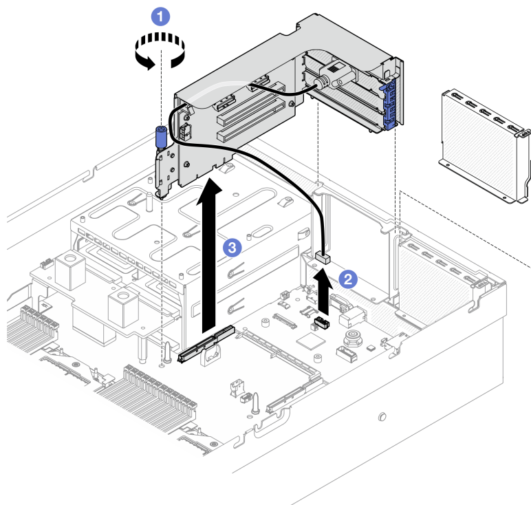
圖例 68. 卸下 PCIe 擴充卡 2 (含序列埠模組)
