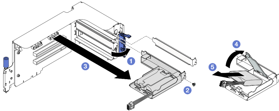
圖例 23. 卸下快閃記憶體電源模組
