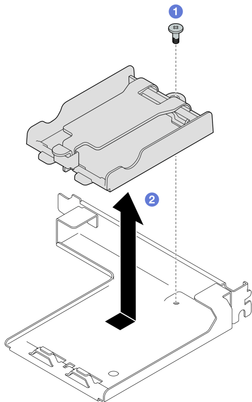
圖例 24. 卸下快閃記憶體電源模組匣
