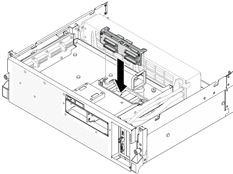
圖例 165. 安裝 2.5 吋硬碟背板模組
