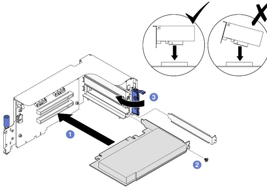
圖例 64. 安裝背面 PCIe 配接卡
