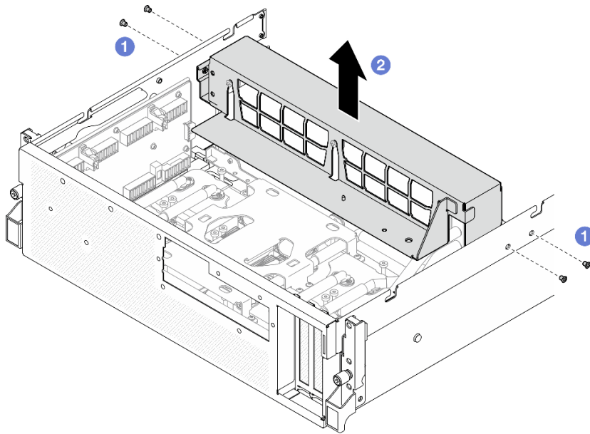
圖例 209. 卸下散熱器托架
