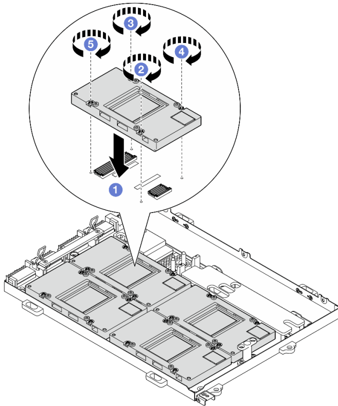
圖例 259. 安裝 SXM5 GPU
