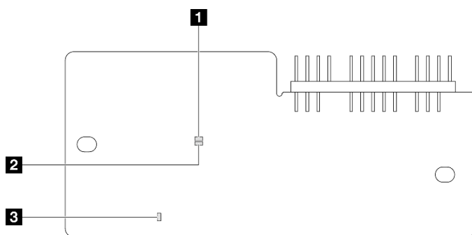
圖例 386. 韌體和 RoT 安全模組上的 LED
