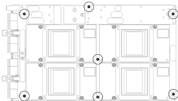
圖例 268. 安裝 1 號十字螺絲
