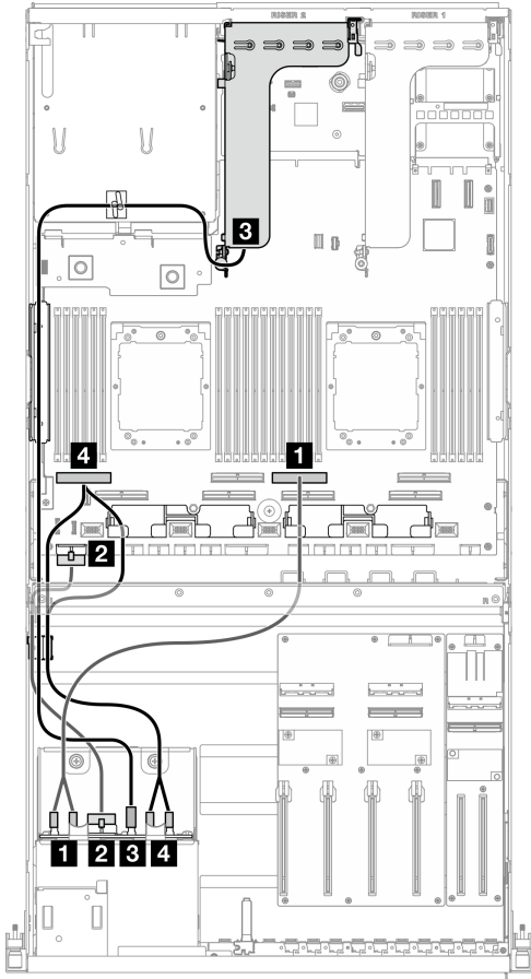
圖例 300. 2.5 吋硬碟背板纜線佈線
