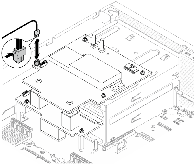
圖例 277. CX-7 支架板電源線連接
