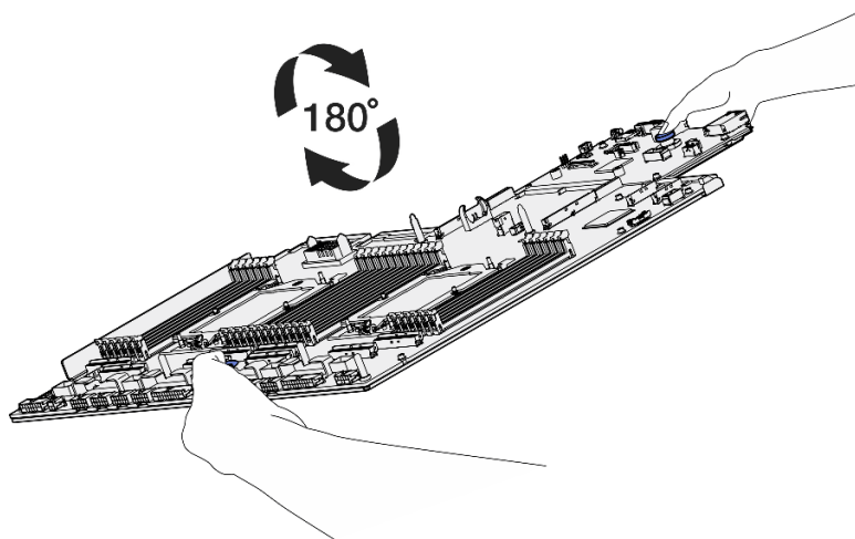
圖例 94. 翻轉主機板組件
