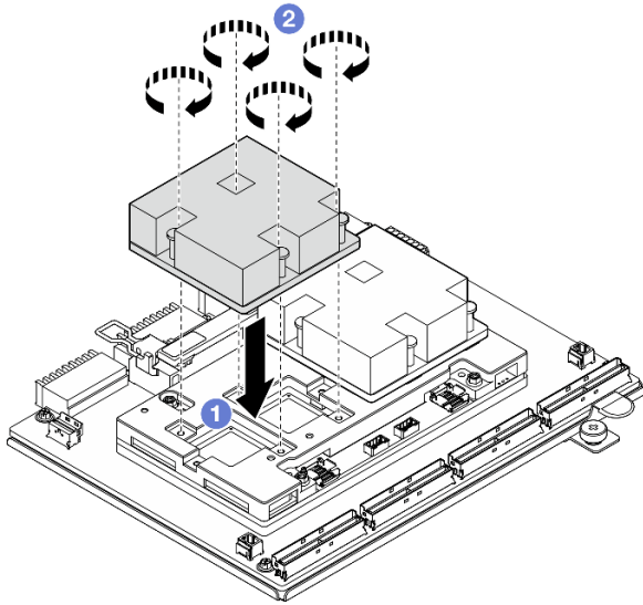
圖例 180. 安裝CX-7 散熱槽
