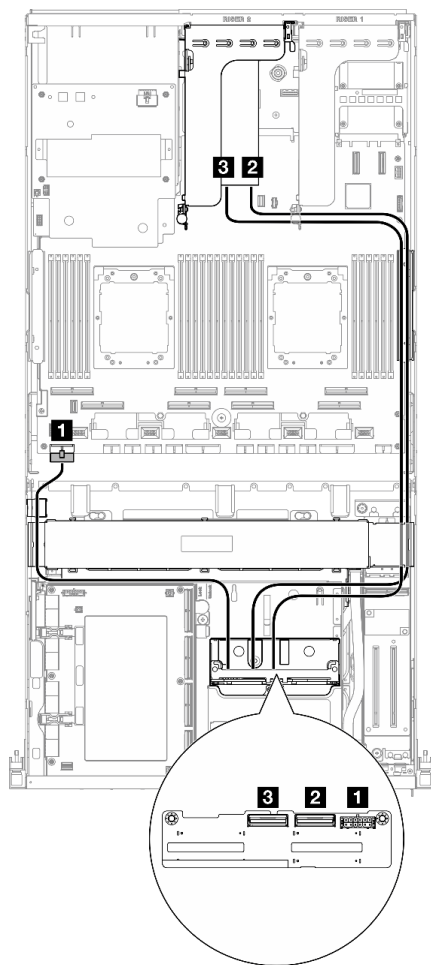
圖例 340. 2.5 吋硬碟背板纜線佈線 (RAID 配接卡在 PCIe 擴充卡 2 上)
