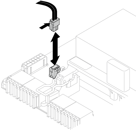
圖例 171. 拔除電源線
