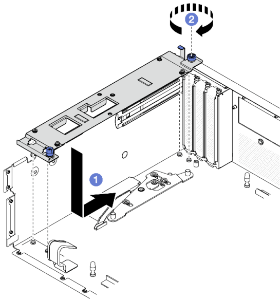
圖例 211. 安裝正面 I/O 擴充板支架
