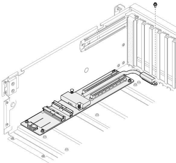
圖例 138. 卸下螺絲
