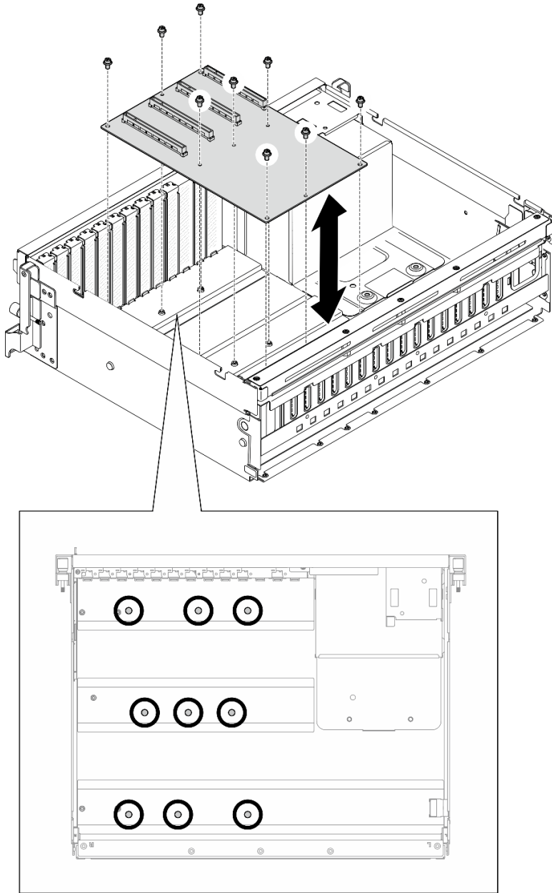
圖例 147. 卸下 GPU 配電板 — 4-DW GPU 型號
