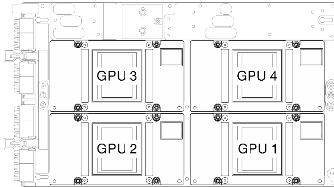
圖例 258. SXM5 GPU 編號
