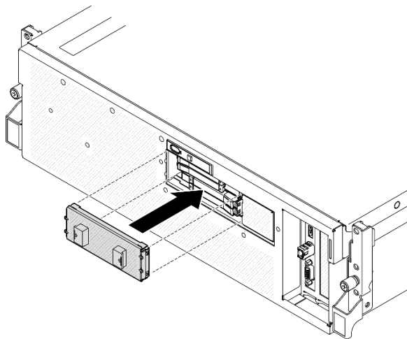
圖例 185. 安裝 E3.S 框架外蓋
