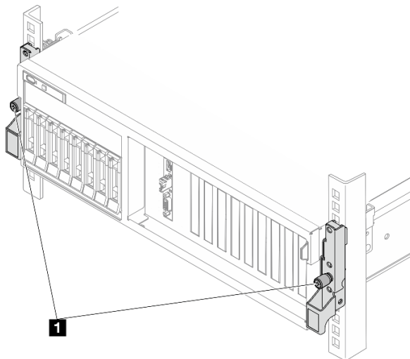
圖例 11. 將伺服器固定到機架正面
