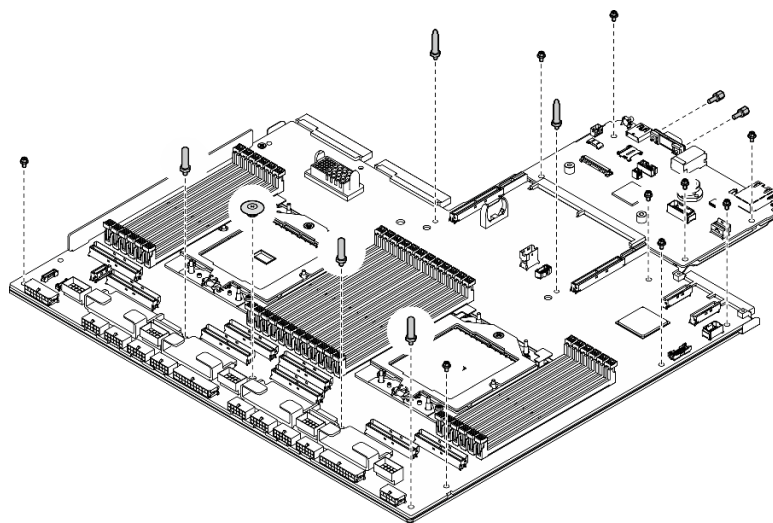
圖例 102. 安裝元件
