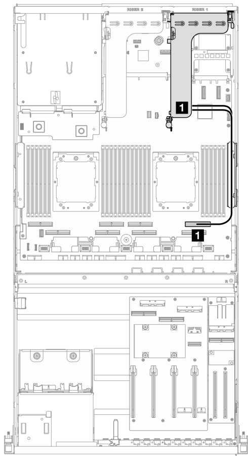
圖例 315. PCIe 擴充卡 1 纜線佈線
