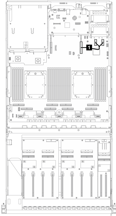
圖例 330. OCP 模組纜線佈線
