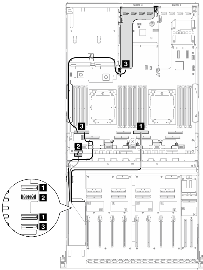
圖例 318. E1.S 硬碟背板纜線佈線
