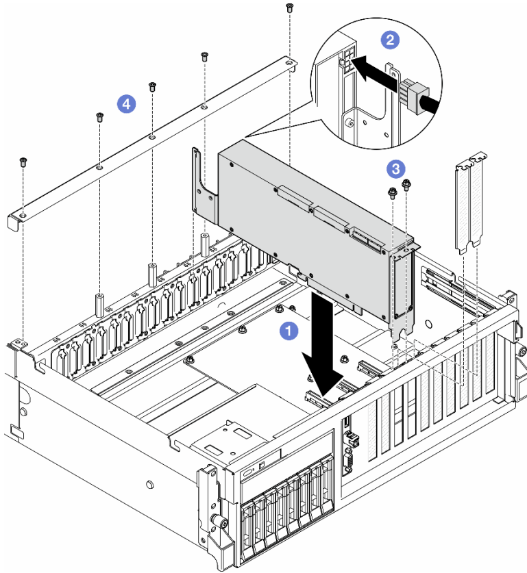
圖例 145. 安裝 GPU 配接卡
