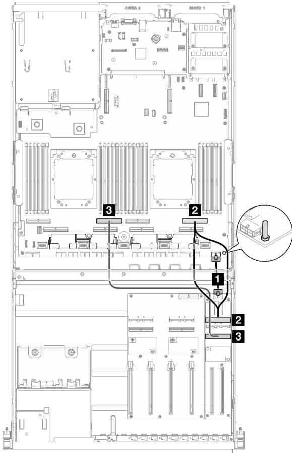
圖例 304. 正面 I/O 擴充板纜線佈線
