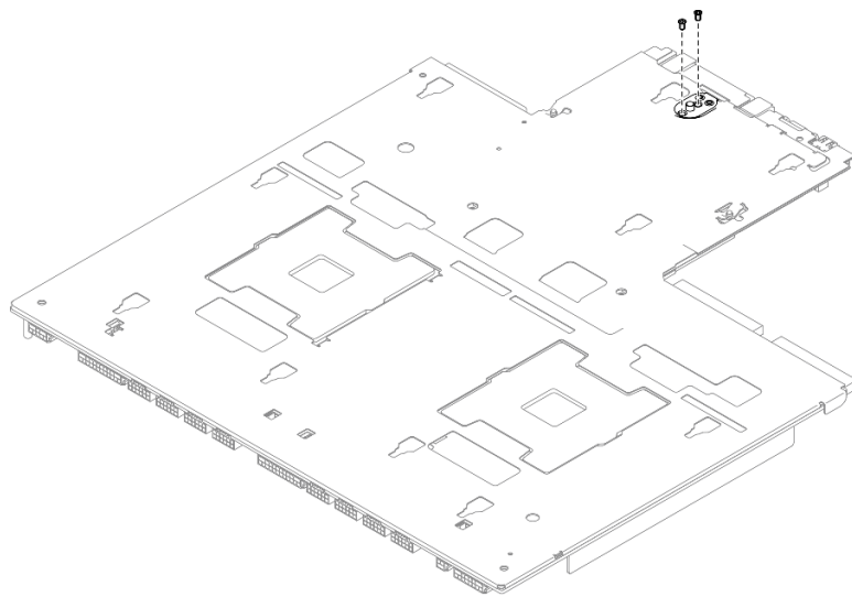
圖例 95. 卸下螺絲
