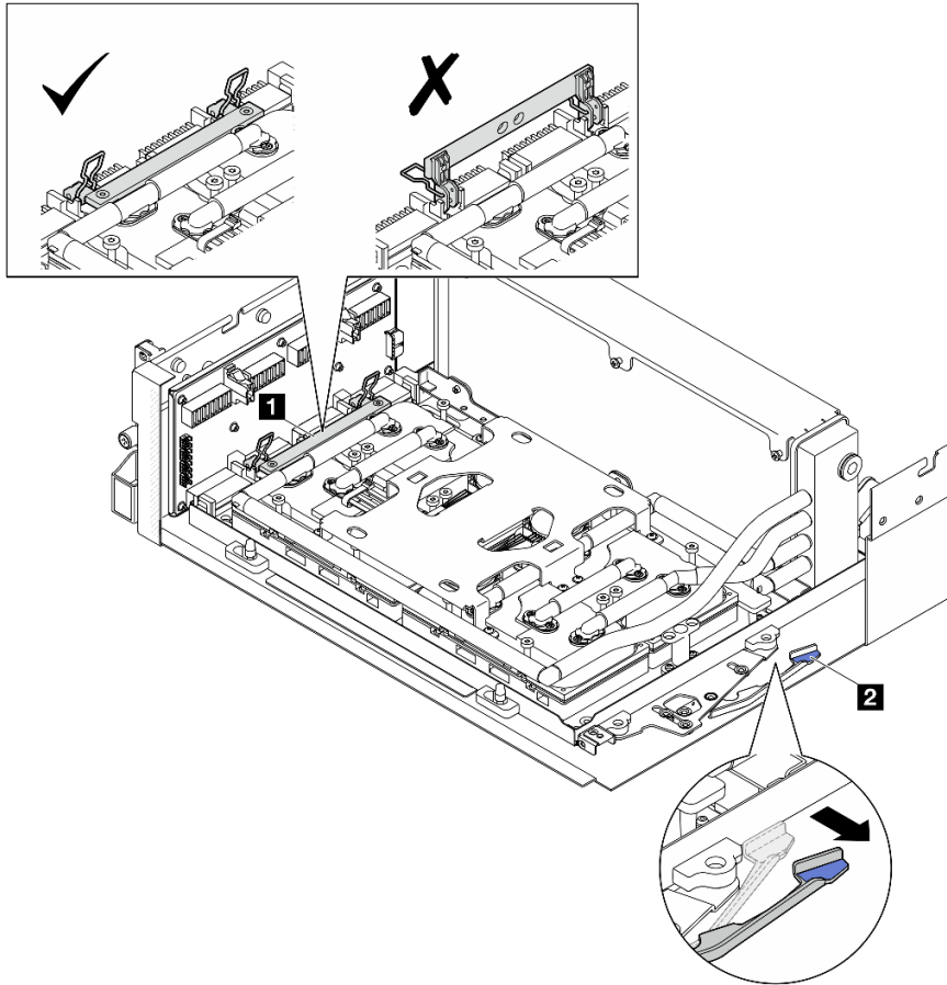
圖例 217. GPU-L2A 組件調整
