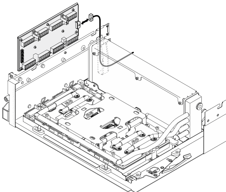
圖例 220. 拔除轉插卡電源線
