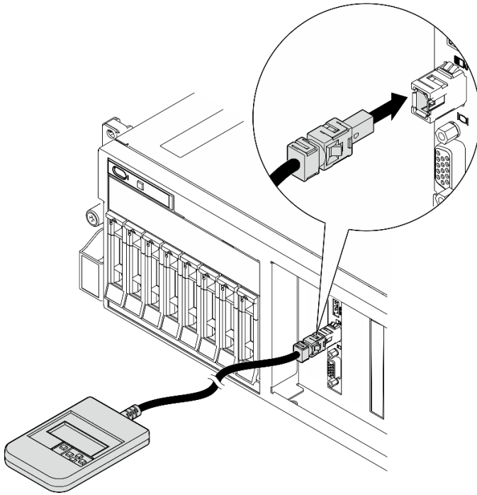
圖例 17. 連接外部診斷手持裝置纜線
