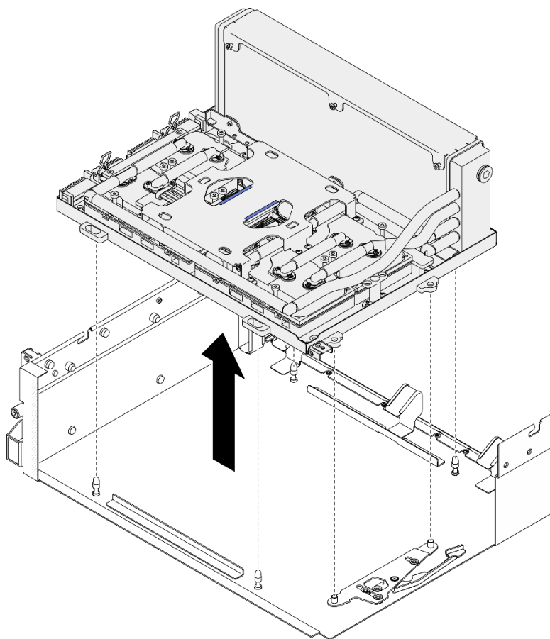
圖例 232. 卸下 GPU-L2A 組件
