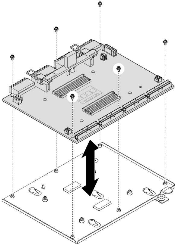
圖例 173. 拆卸 CX-7 支架板
