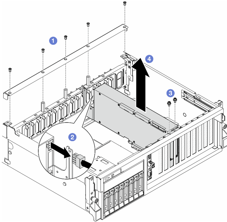
圖例 142. 卸下 GPU 配接卡
