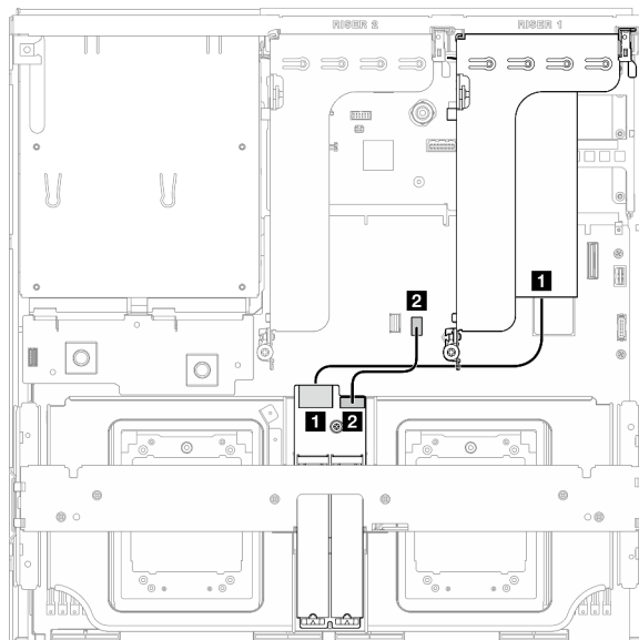
圖例 328. SATA/x4 NVMe M.2 背板纜線佈線 (RAID 配接卡在 PCIe 擴充卡 1 上)
