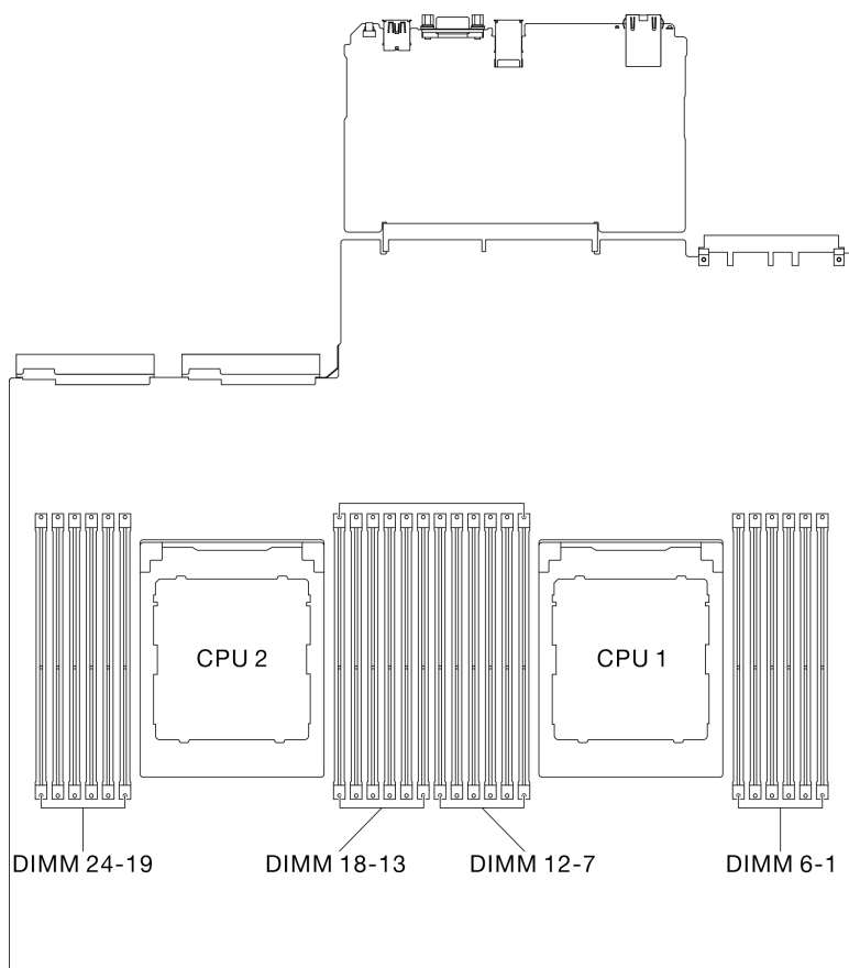
圖例 1. 記憶體模組和處理器佈置
