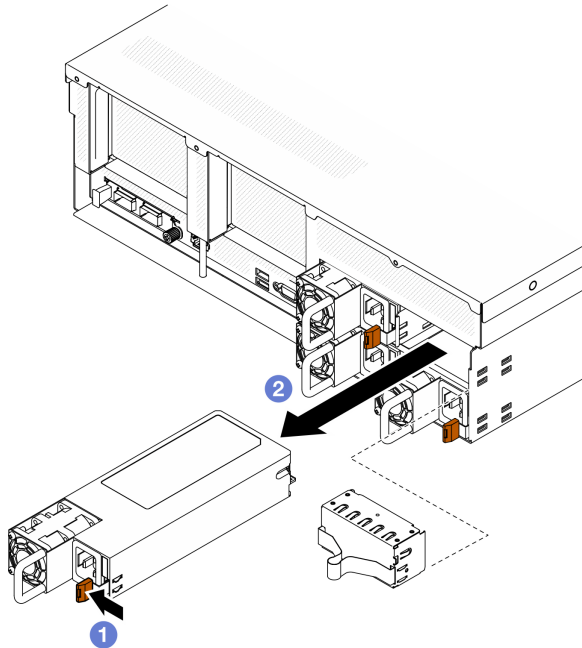
圖例 77. 電源供應器卸下
