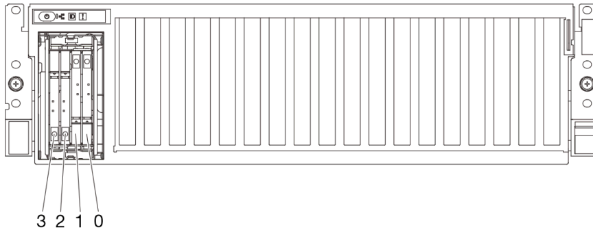
圖例 123. 8-DW GPU 型號中的 E3.S 熱抽換機槽編號
