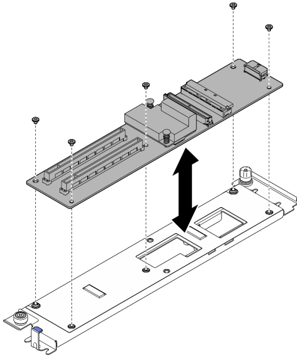
圖例 204. 安裝正面 I/O 擴充板
