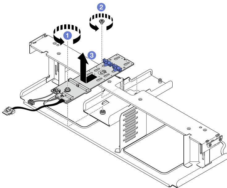
圖例 40. 卸下 M.2 背板
