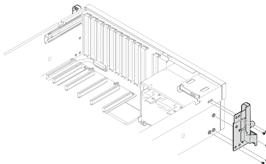
圖例 56. 卸下左安裝把手
