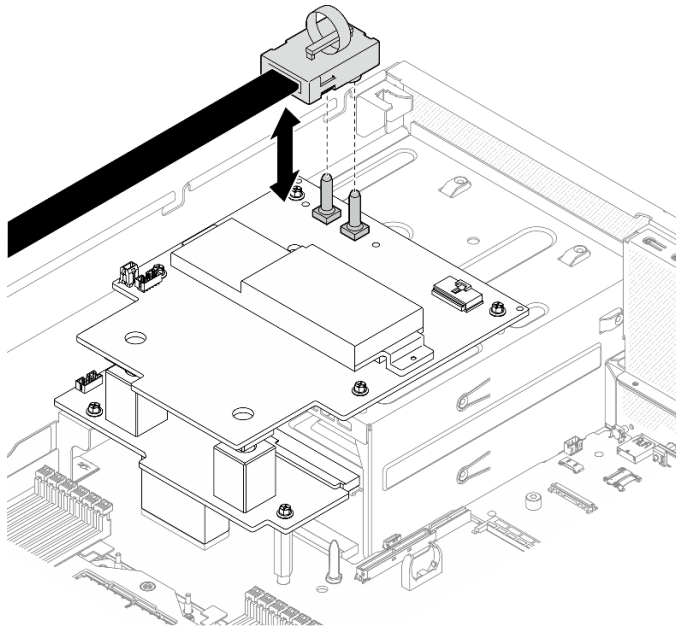
圖例 271. 拔除 SXM5 GPU 板組件電源線
