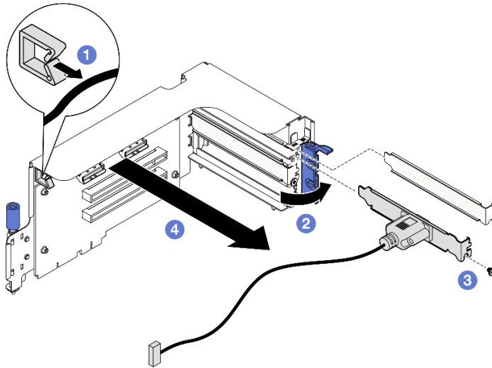
圖例 86. 卸下序列埠模組
