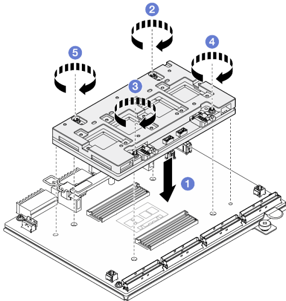
圖例 174. 安裝 CX-7 Mezz 板
