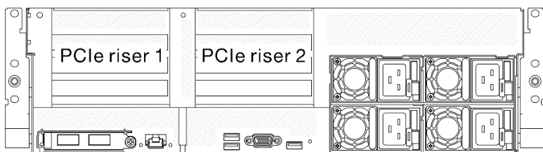
圖例 69. PCIe 擴充卡位置
