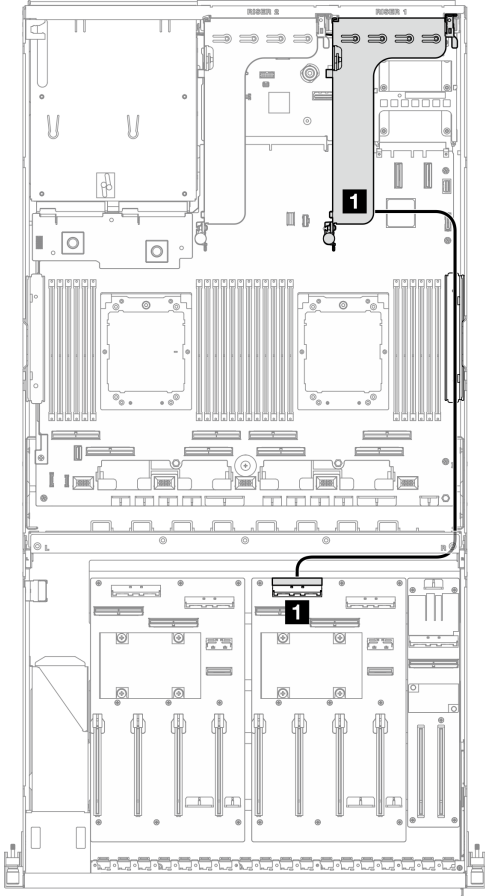
圖例 333. PCIe 擴充卡 1 纜線佈線
