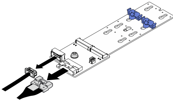
圖例 44. 連接 SATA/x4 NVMe M.2 背板纜線
