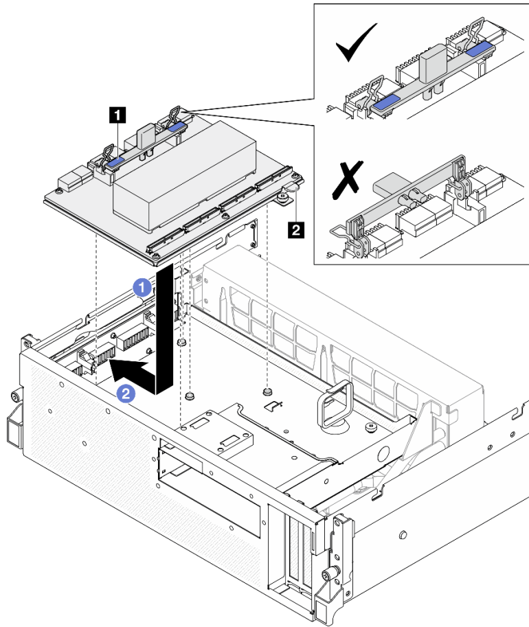
圖例 282. 安裝 SXM5 PCIe 交換器板
