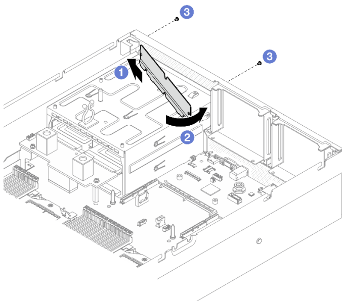
圖例 159. 安裝熱氣流後擋板
