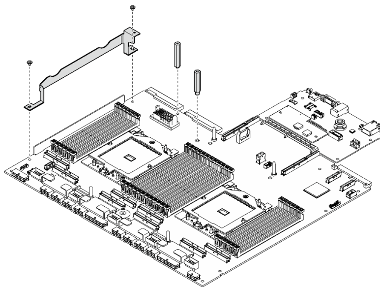
圖例 106. 安裝元件
