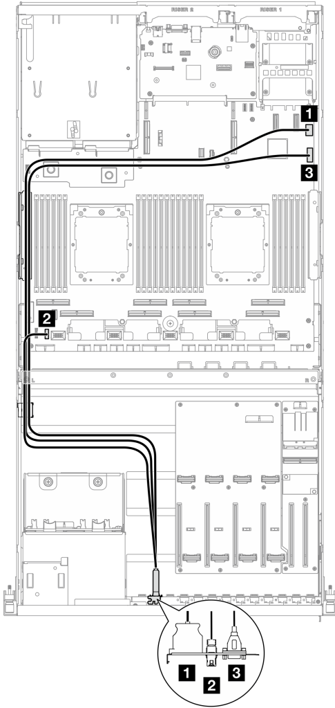
圖例 28. 正面 I/O 模組的纜線佈線 — 4-DW GPU 型號
