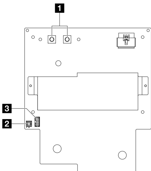
圖例 295. SXM5 GPU 電源配送板接頭
