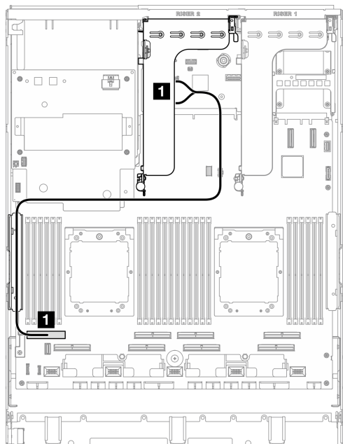
圖例 372. PCIe 擴充卡 2 纜線佈線
