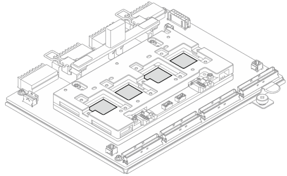
圖例 178. 擦掉 ASIC 上的油灰墊
