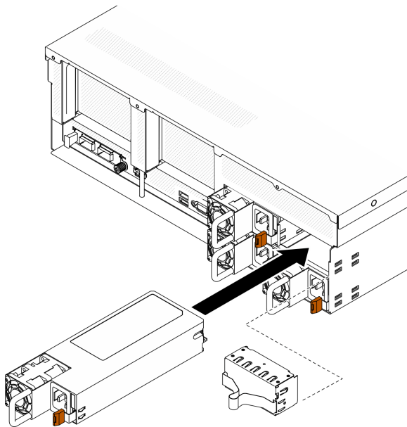
圖例 79. 安裝電源供應器
