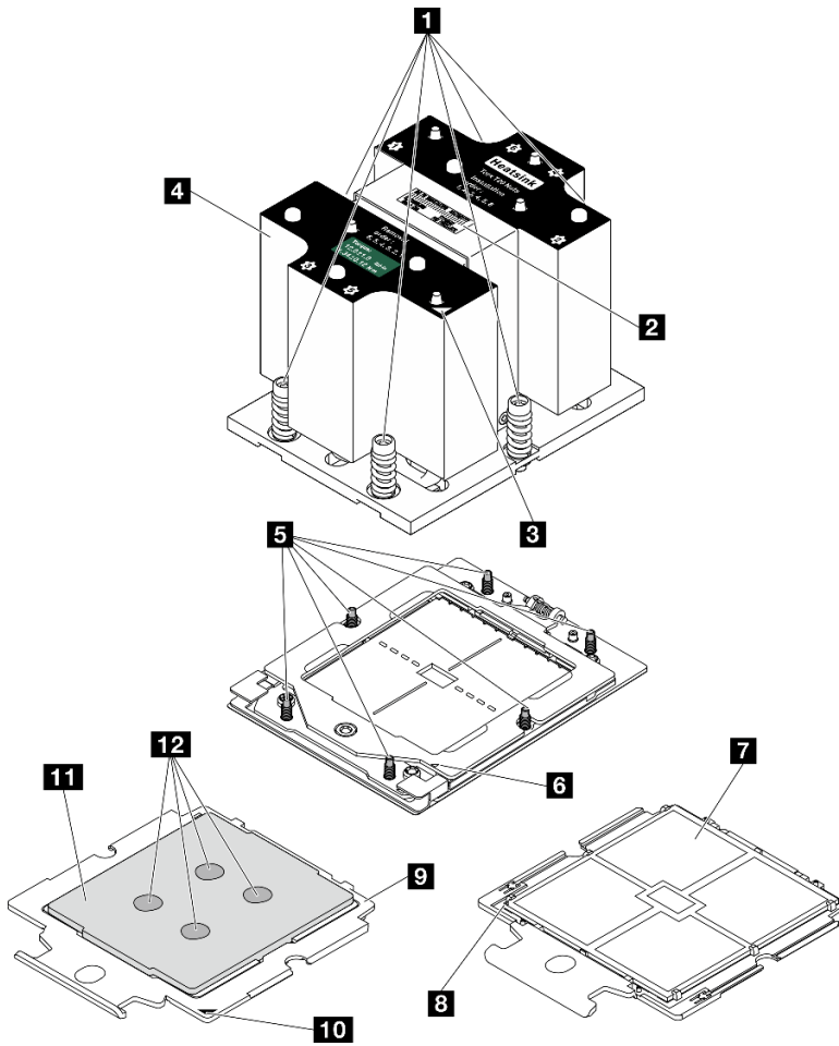
圖例 80. 處理器和散熱槽元件
