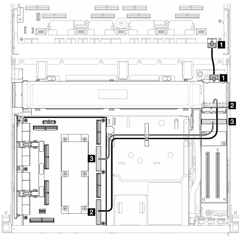
圖例 358. 正面 I/O 擴充板纜線佈線
