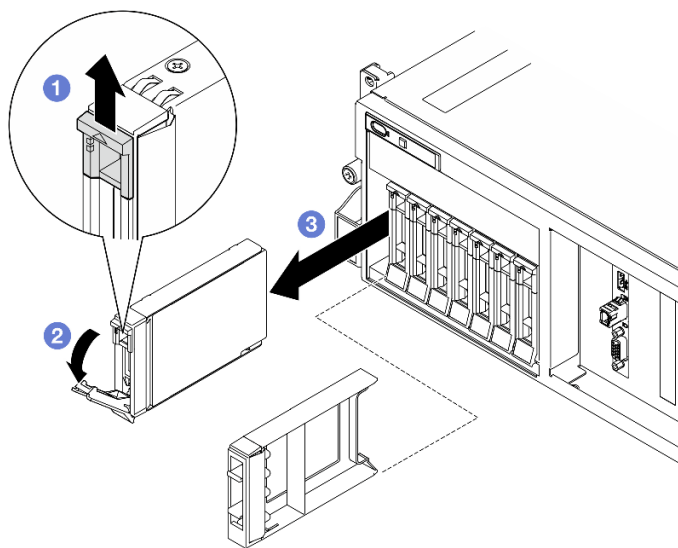
圖例 111. 卸下 2.5 吋熱抽換硬碟
