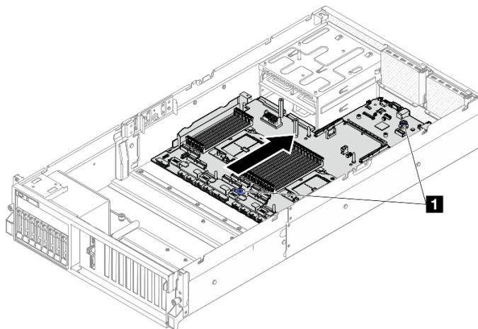
圖例 108. 安裝主機板組件
