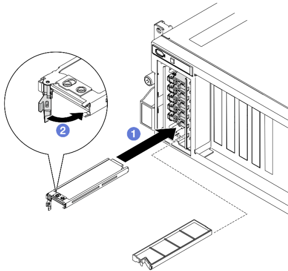
圖例 125. 安裝 E1.S 熱抽換硬碟
