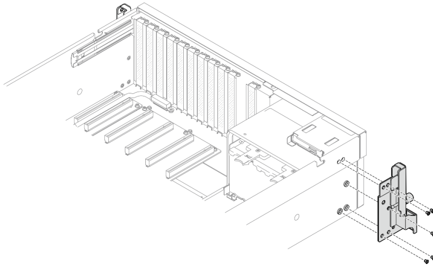
圖例 58. 安裝左安裝把手
