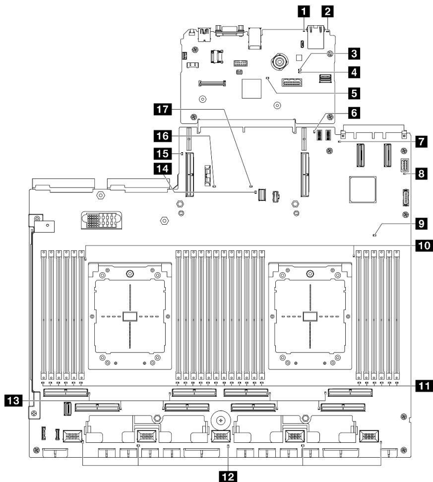
圖例 385. 主機板組件 LED
