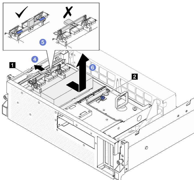
圖例 279. 卸下 SXM5 PCIe 交換器板
