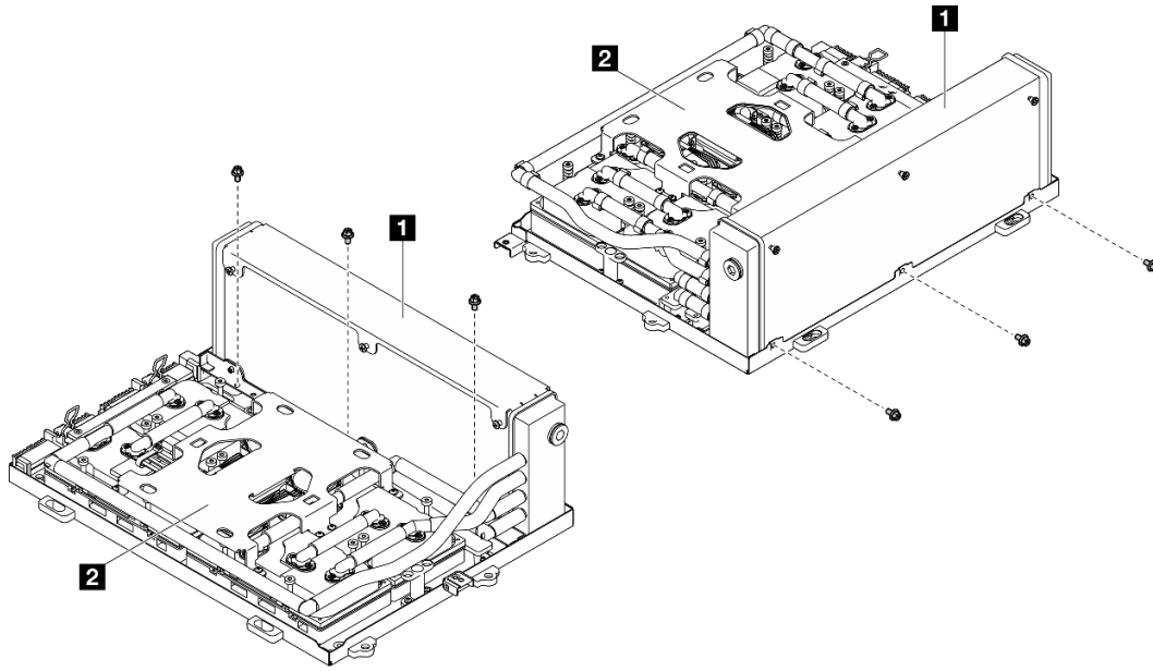
圖例 233. 卸下 1 號十字螺絲
