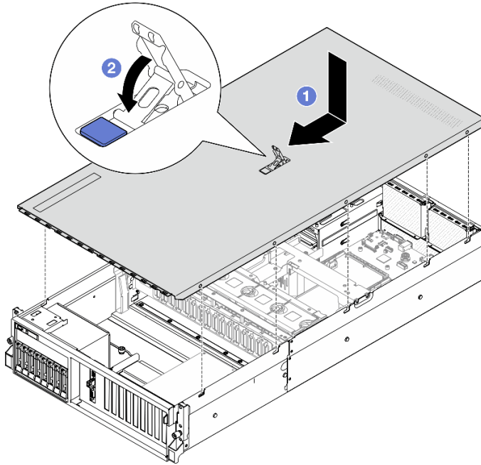
圖例 110. 安裝上蓋
