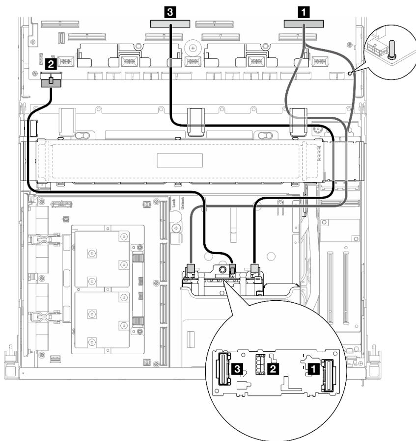
圖例 356. E3.S 硬碟背板纜線佈線
