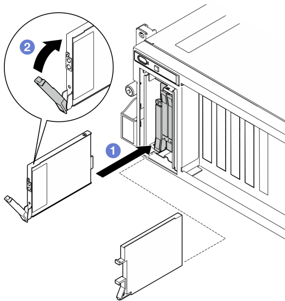
圖例 126. 安裝 E3.S 熱抽換硬碟
