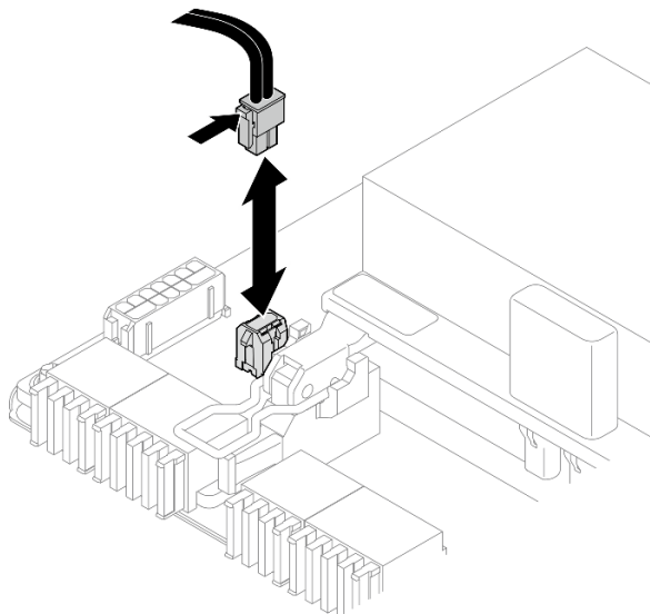
圖例 175. 拔除電源線
