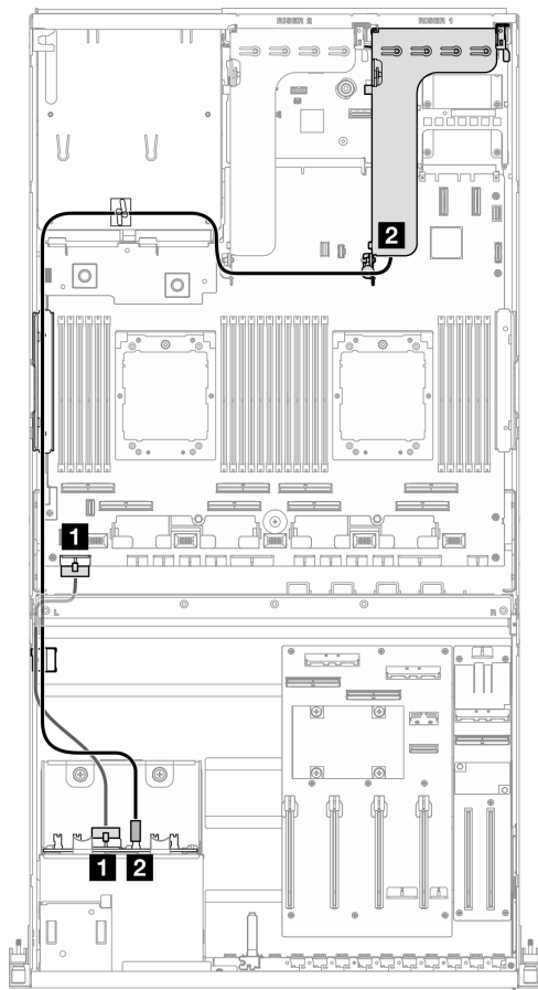
圖例 301. 2.5 吋硬碟背板纜線佈線
