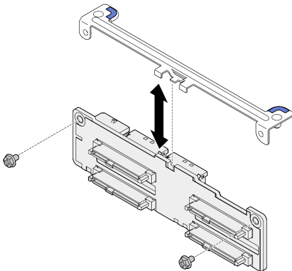
圖例 164. 卸下 2.5 吋硬碟背板托架
