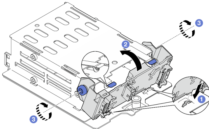
圖例 189. 安裝 E3.S 硬碟背板模組
