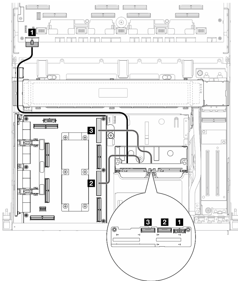
圖例 338. 2.5 吋硬碟背板纜線佈線
