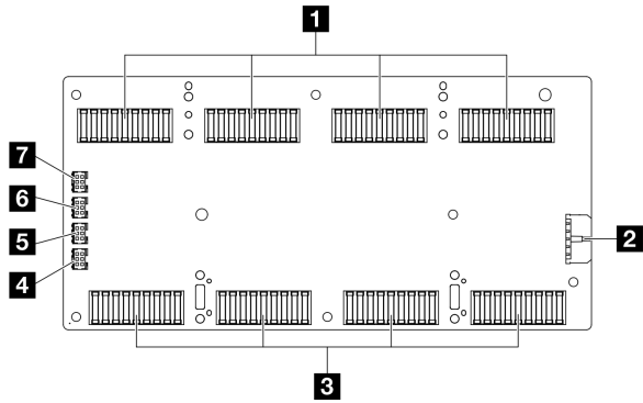
圖例 292. 轉插卡接頭
