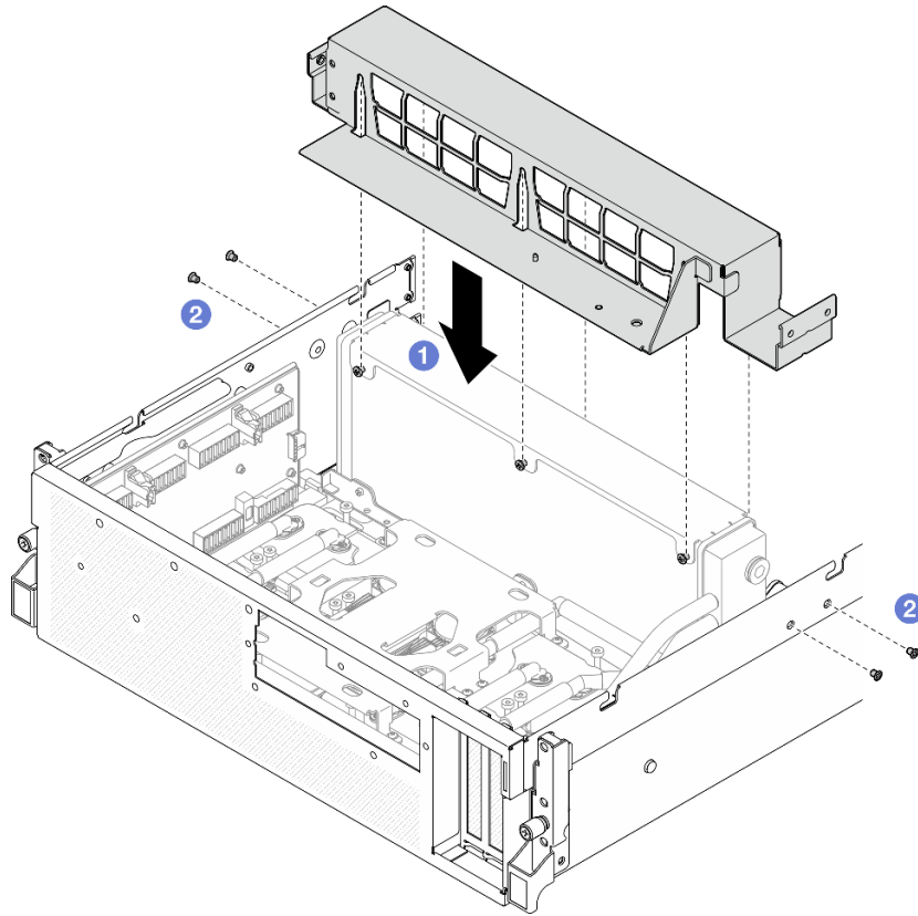
圖例 206. 安裝散熱器托架
