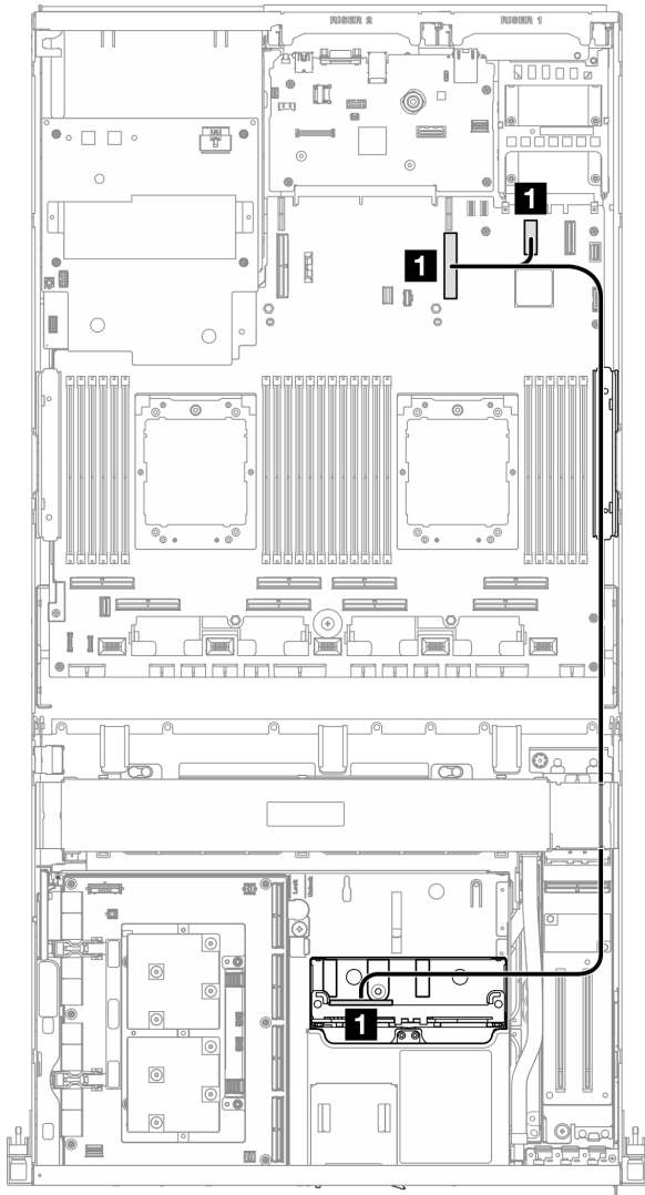
圖例 365. OCP 模組纜線佈線
