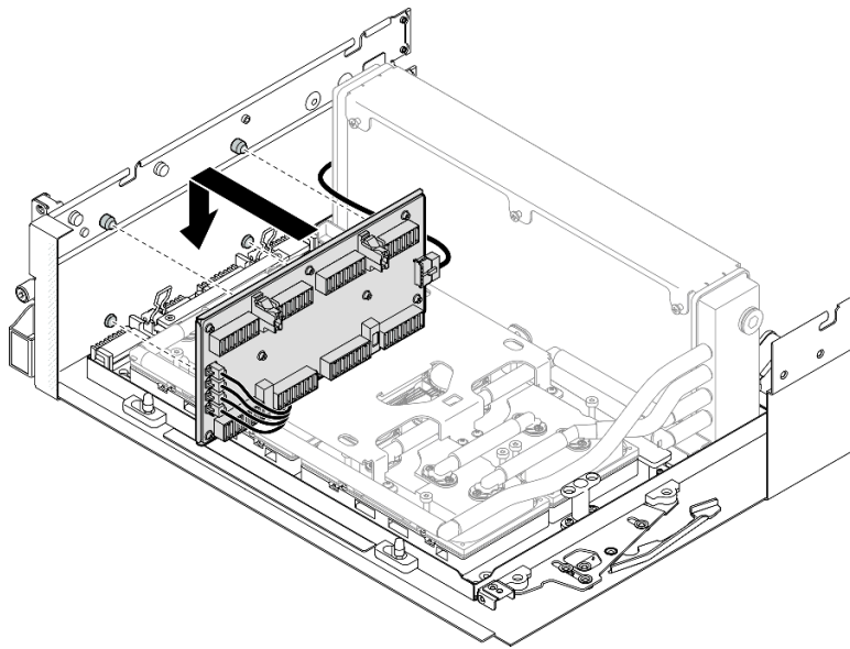
圖例 225. 轉插卡安裝
