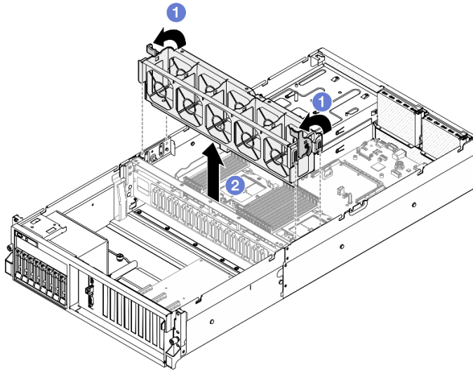
圖例 21. 卸下風扇機盒
