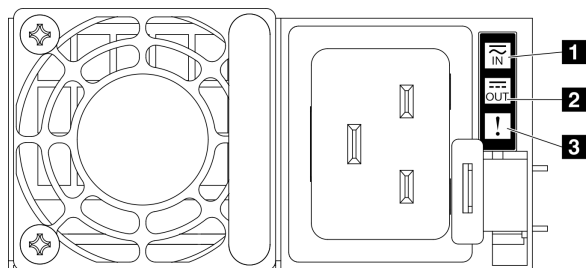
圖例 383. 電源供應器 LED
