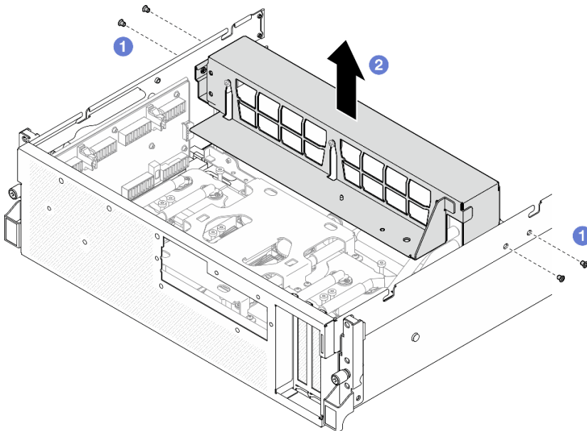
圖例 201. 卸下散熱器托架
