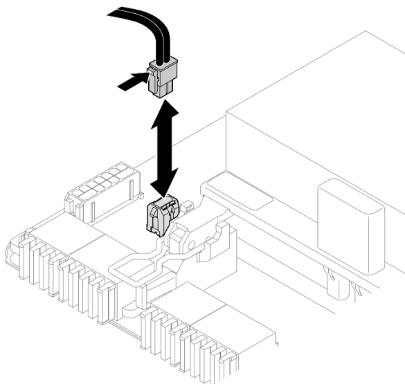
圖例 168. 拔除電源線
