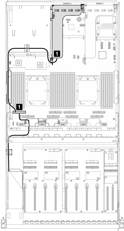
圖例 335. PCIe 擴充卡 2 纜線佈線
