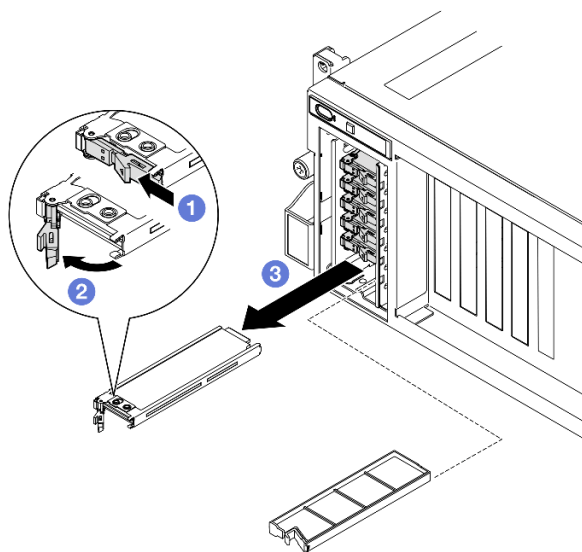
圖例 119. 卸下 E1.S 熱抽換硬碟
