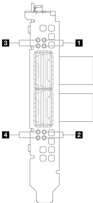
圖例 382. OSFP 埠卡 LED
