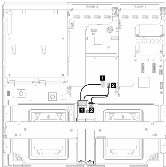
圖例 361. SATA/NVMe 或 NVMe RAID M.2 背板纜線佈線
