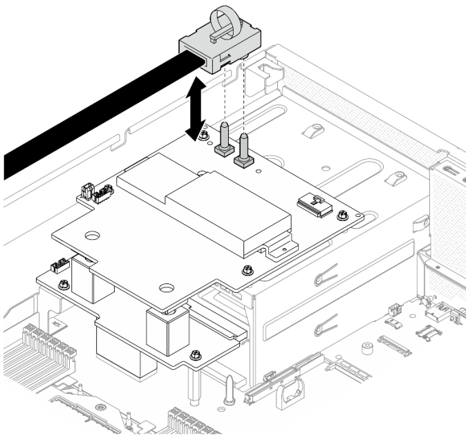
圖例 278. SXM5 GPU 板組件電源線連接
