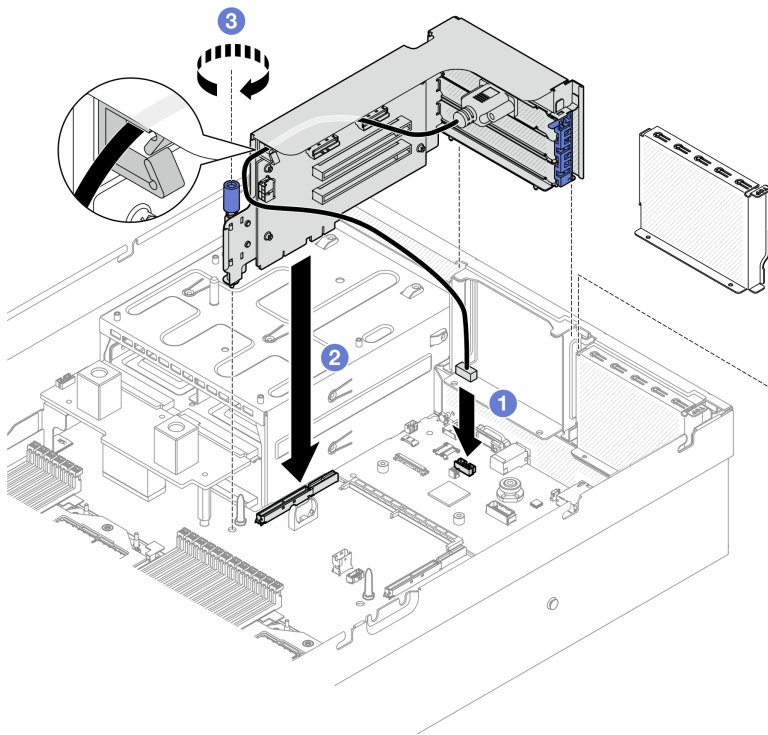
圖例 72. 安裝 PCIe 擴充卡 2 (含序列埠模組)
