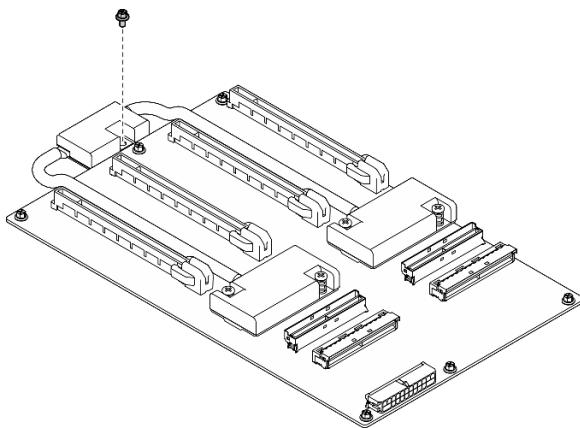
圖例 146. 卸下螺絲
