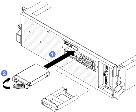
圖例 162. 安裝 2.5 吋熱抽換硬碟
