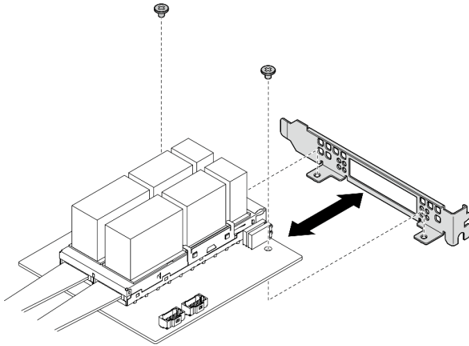
圖例 252. 拆卸 OSFP 埠卡
