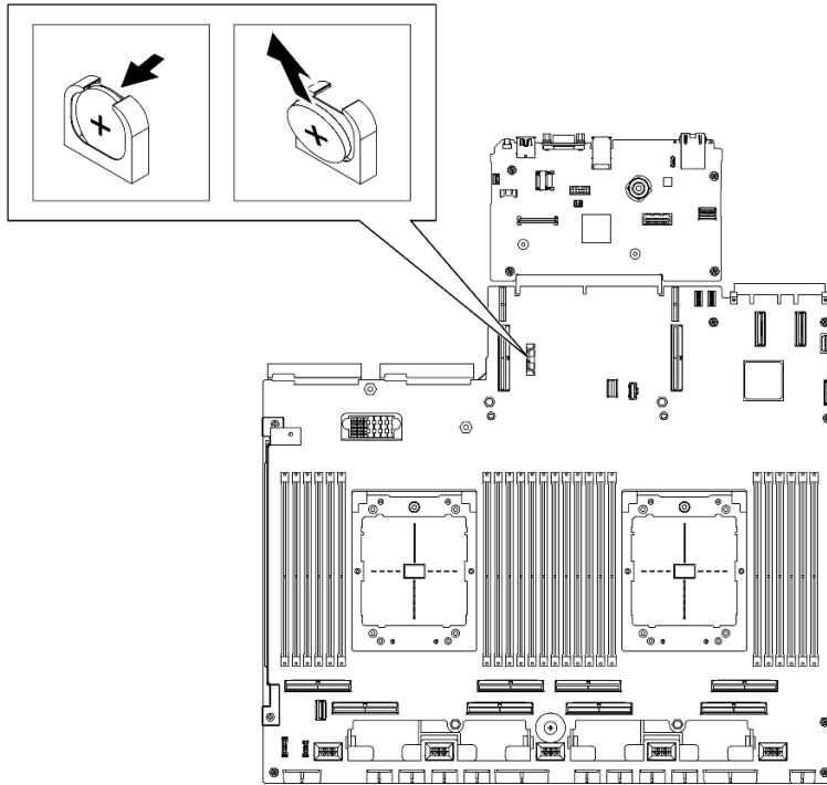
圖例 14. 卸下 CMOS 電池
