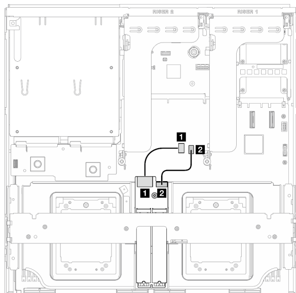
圖例 360. SATA/x4 NVMe M.2 背板纜線佈線
