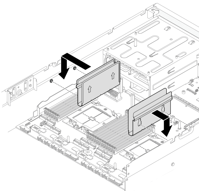
圖例 52. 安裝纜線導件
