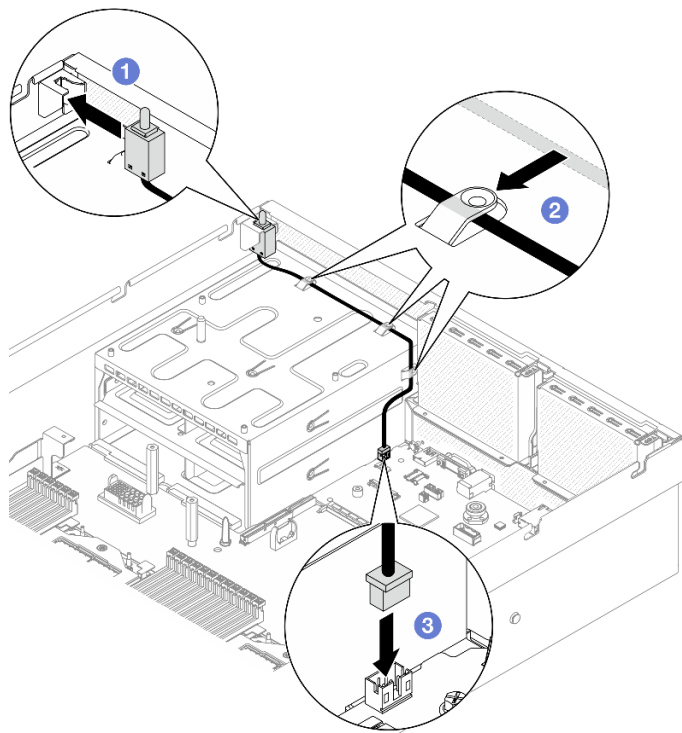
圖例 37. 入侵開關安裝
