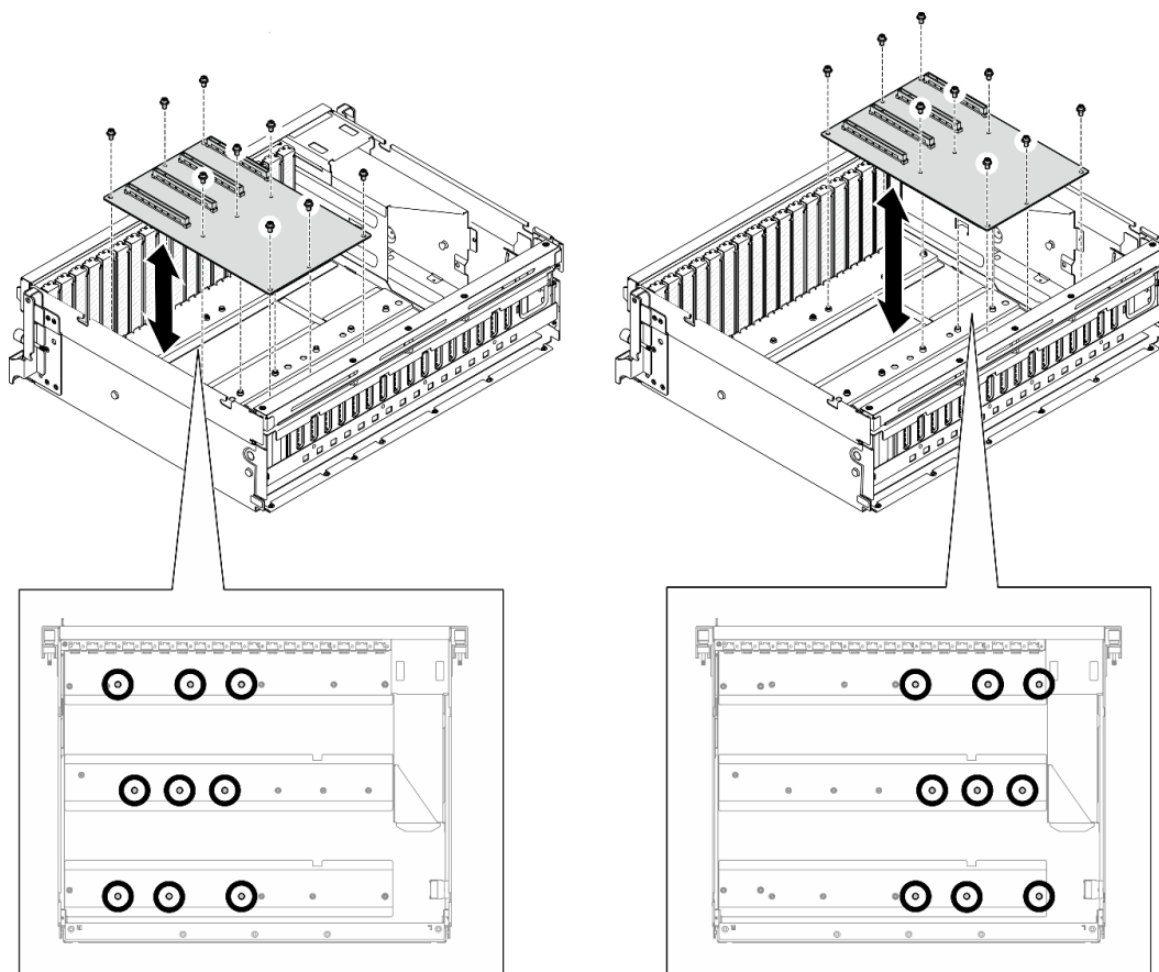
圖例 148. 卸下 GPU 配電板 — 8-DW GPU 型號
