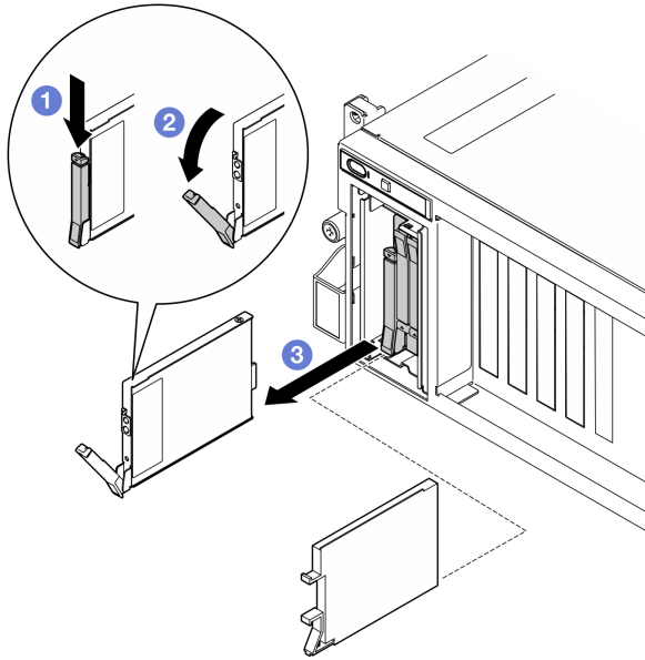
圖例 120. 卸下 E3.S 熱抽換硬碟
