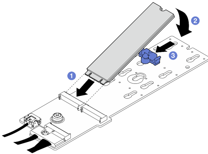
圖例 46. M.2 硬碟安裝
