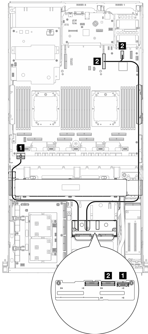
圖例 343. 2.5 吋硬碟背板纜線佈線
