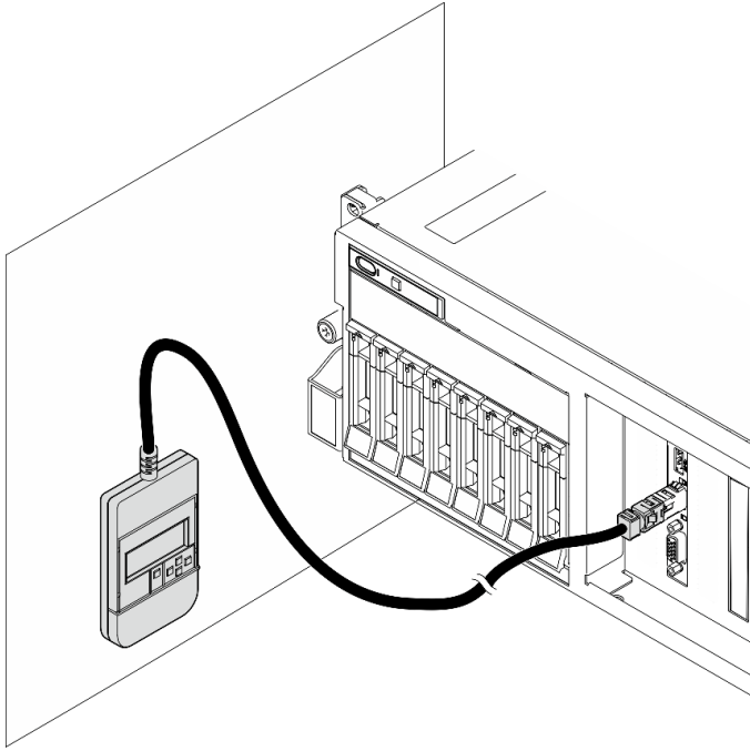
圖例 18. 將外部診斷手持裝置連接到金屬表面
