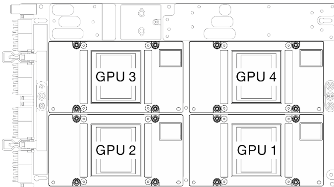
圖例 255. SXM5 GPU 編號
