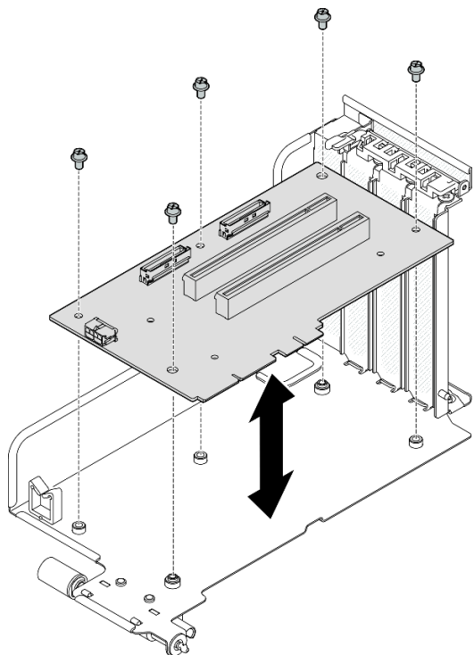
圖例 74. 安裝 PCIe 擴充卡
