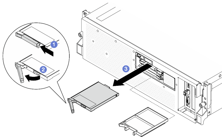
圖例 181. 卸下 E3.S 熱抽換硬碟
