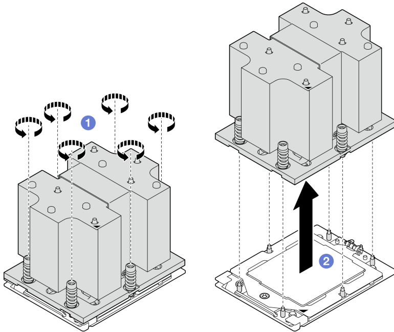
圖例 81. 卸下散熱槽
