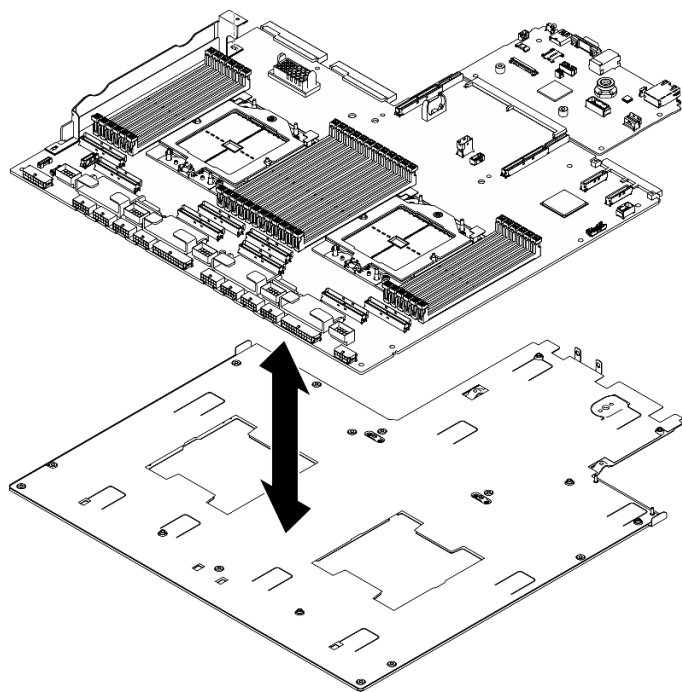
圖例 101. 安裝主機板組件
