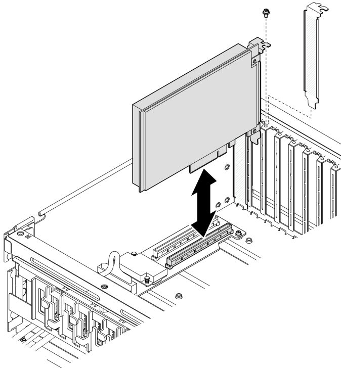
圖例 61. 卸下正面 PCIe 配接卡
