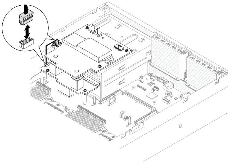
圖例 276. 側頻纜線連接
