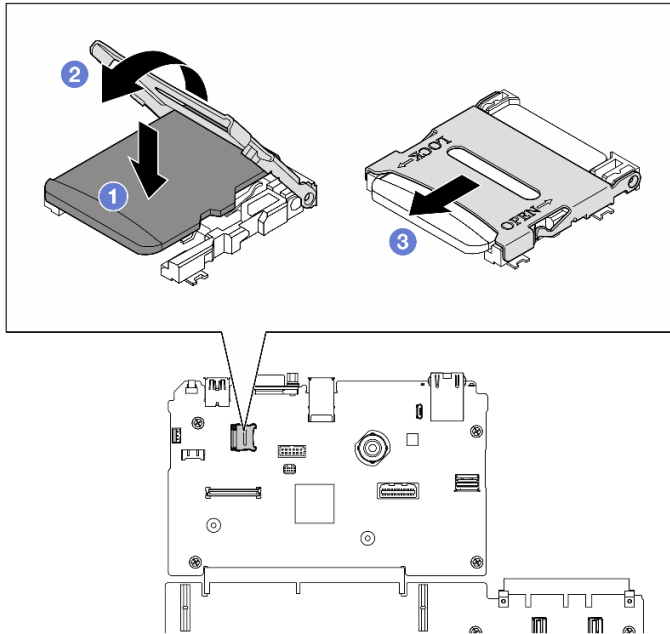
圖例 54. 安裝 MicroSD 卡
