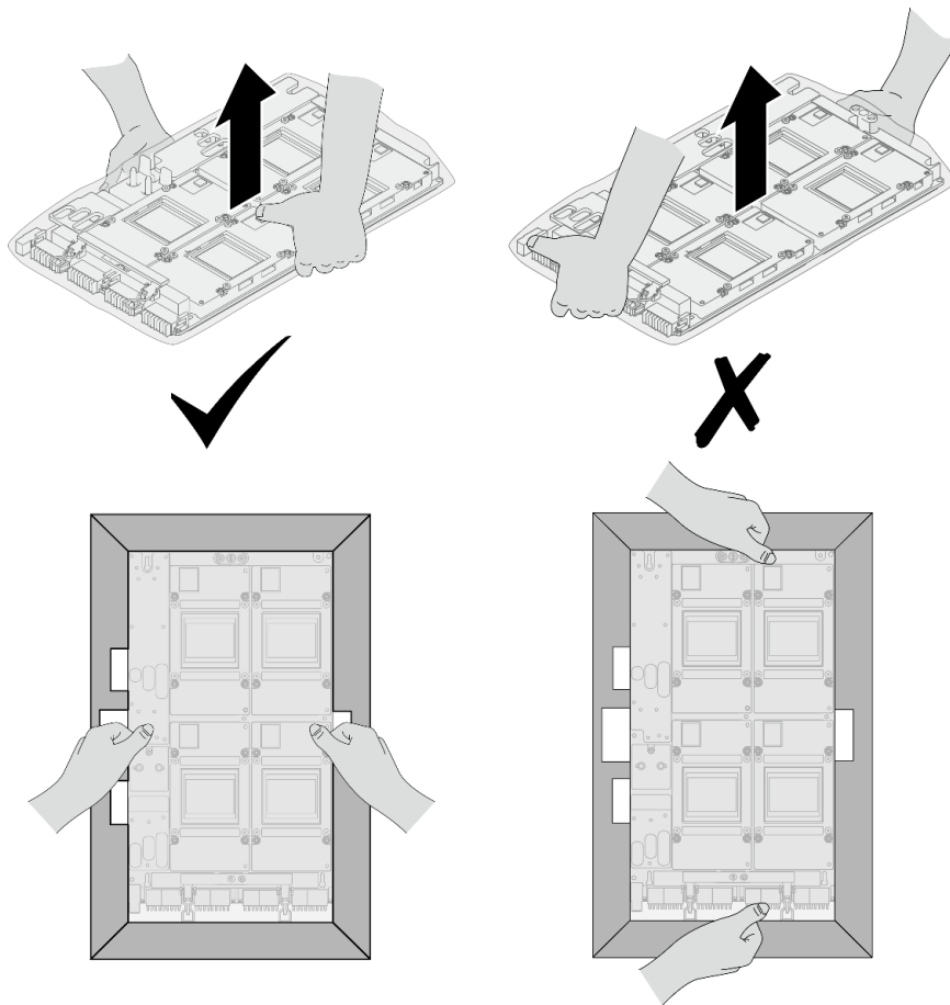
圖例 265. 從包裝盒取出 SXM5 GPU 板組件
