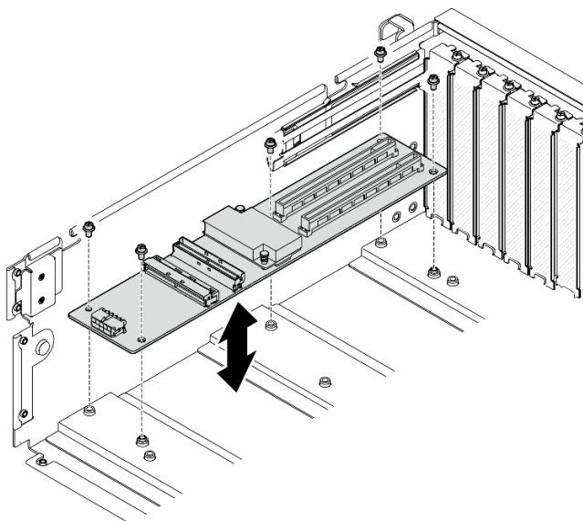
圖例 139. 卸下正面 I/O 擴充板
