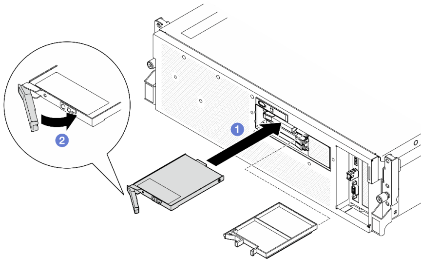
圖例 184. 安裝 E3.S 熱抽換硬碟
