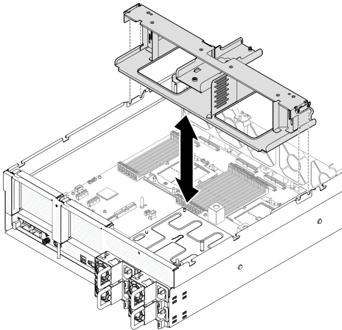
圖例 13. 安裝空氣擋板
