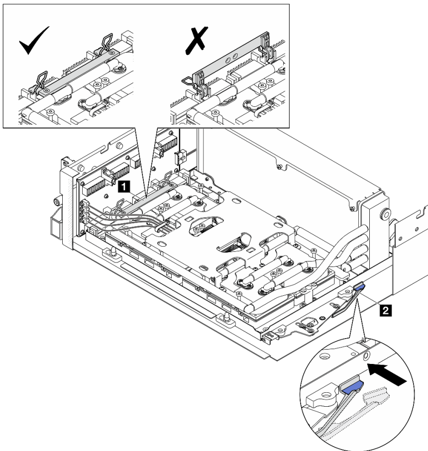
圖例 226. GPU-L2A 組件調整
