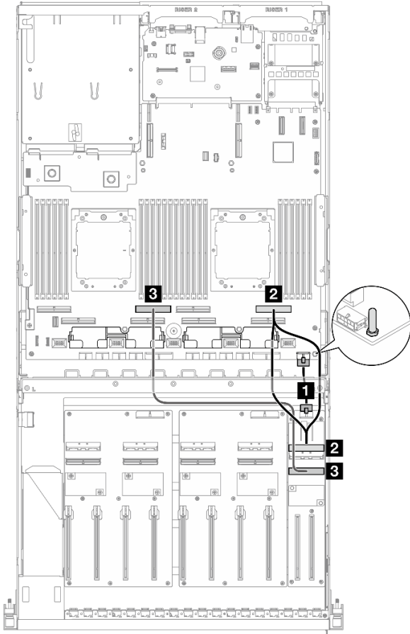
圖例 322. 正面 I/O 擴充板纜線佈線
