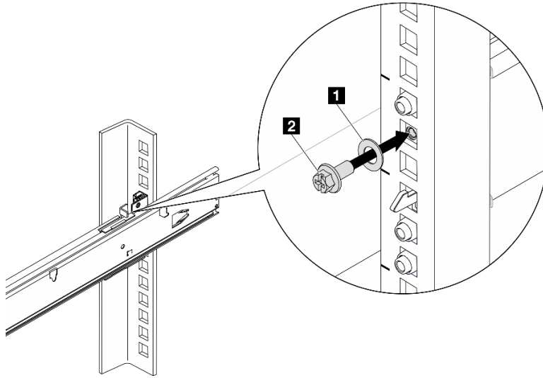
圖例 10. 將伺服器固定到機架背面
