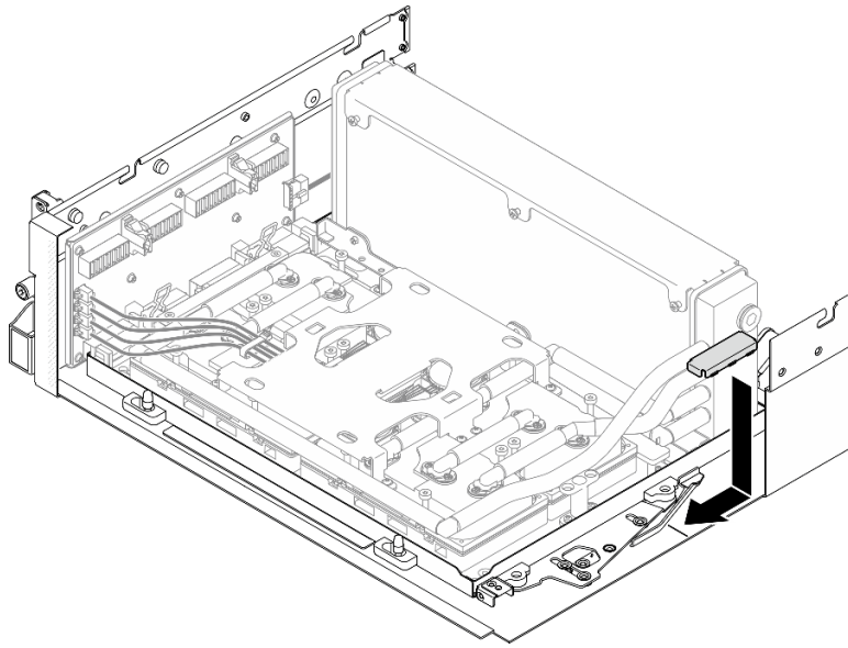
圖例 227. 安裝 SXM5 GPU 板組件固定托架
