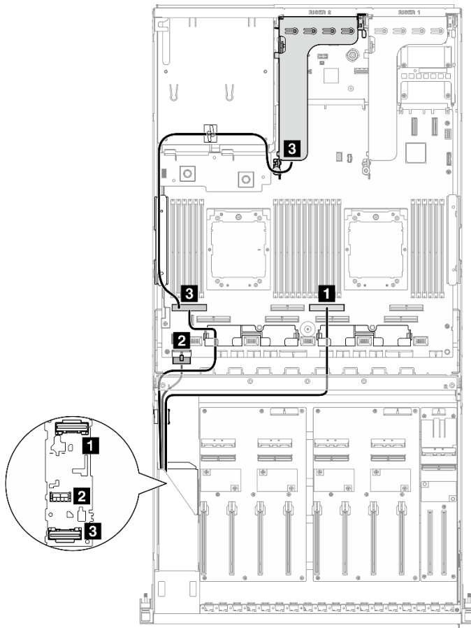
圖例 320. E3.S 硬碟背板纜線佈線
