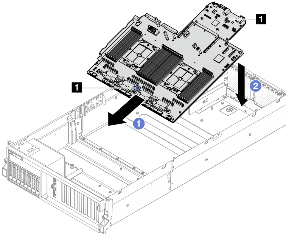
圖例 107. 安裝主機板組件
