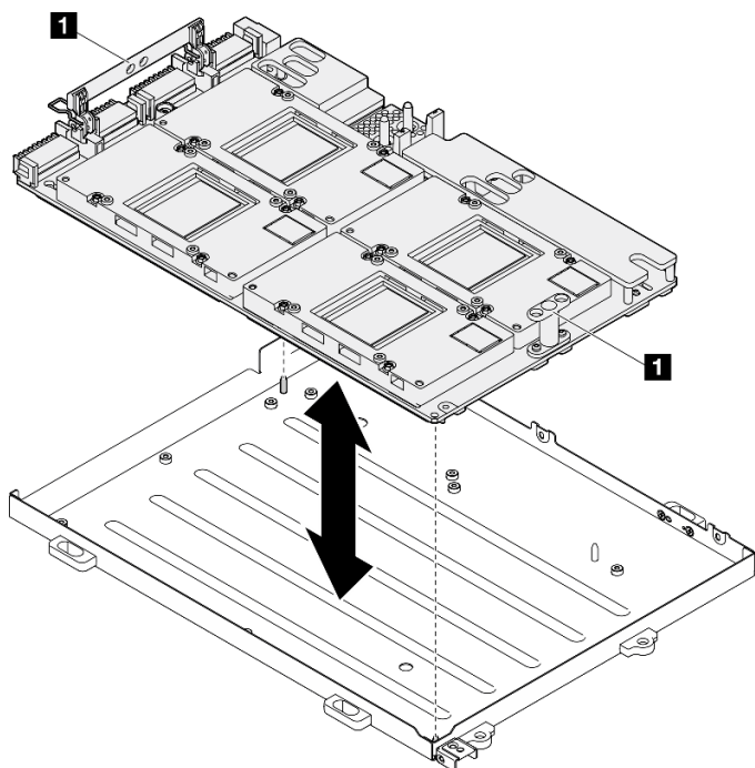
圖例 264. 卸下 SXM5 GPU 板組件
