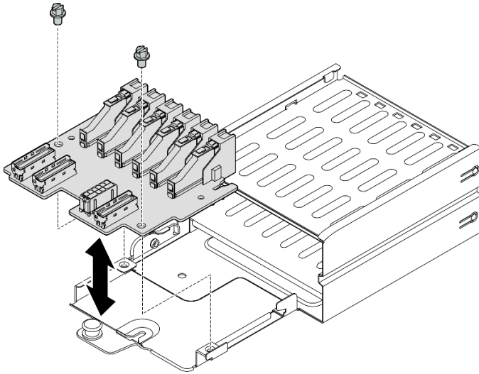
圖例 128. 卸下 E1.S 硬碟背板
