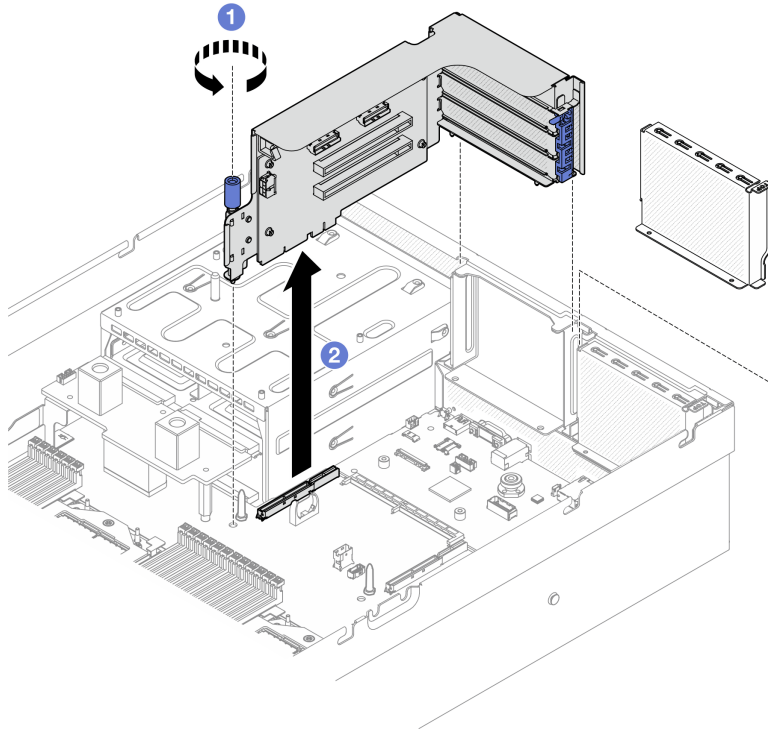
圖例 66. 卸下 PCIe 擴充卡 (不含序列埠模組)
