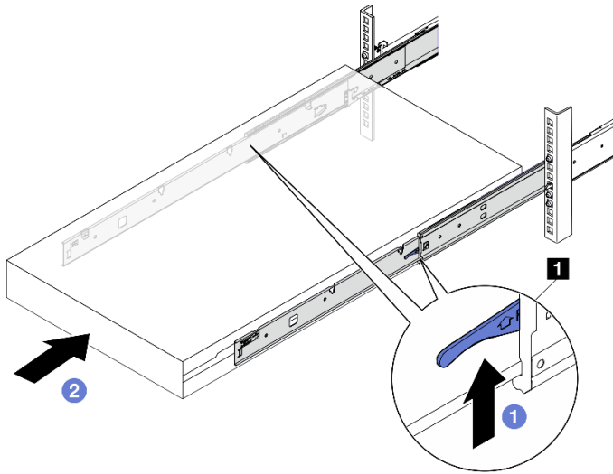
圖例 9. 將伺服器安裝到機架中
