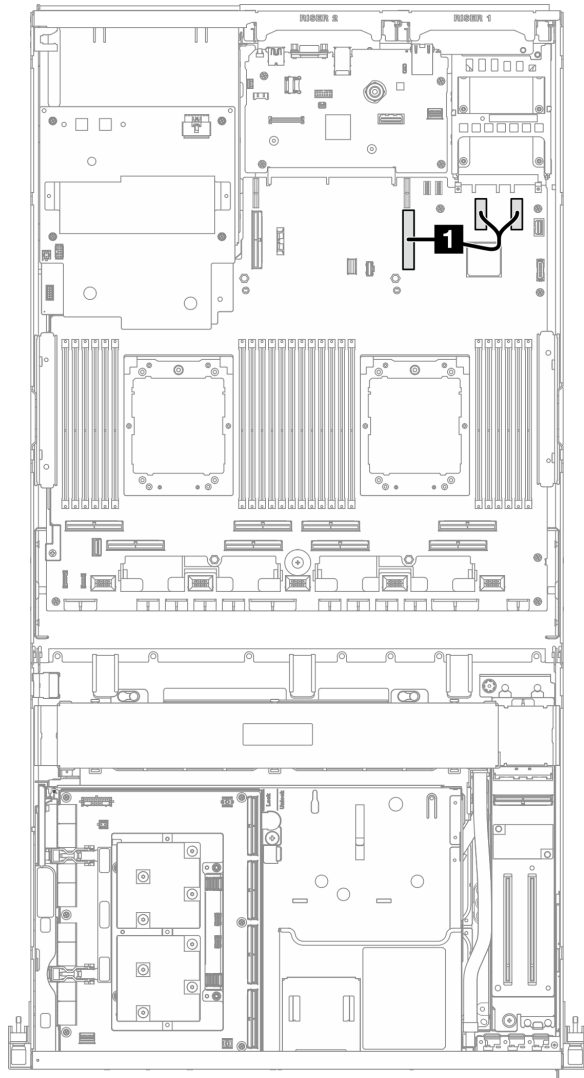
圖例 367. OCP 模組纜線佈線
