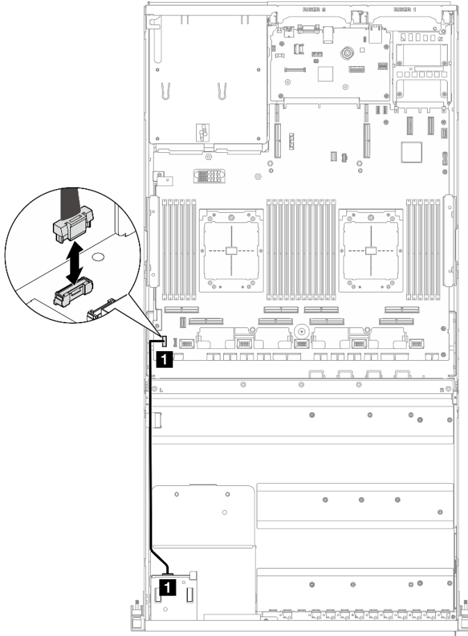
圖例 30. 拔除前方操作面板纜線 — 4-DW GPU 型號和 8-DW GPU 型號
