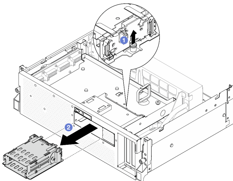
圖例 190. 卸下 E3.S 框架組件
