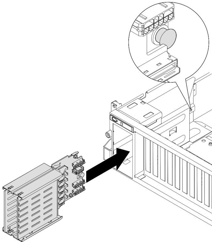
圖例 136. E1.S 框架組件安裝
