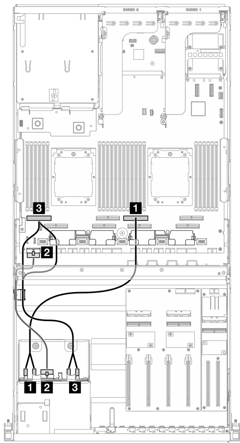
圖例 299. 2.5 吋硬碟背板纜線佈線
