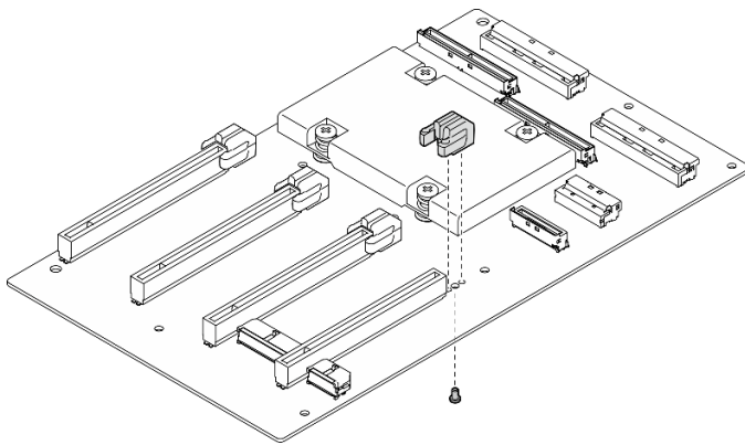
圖例 157. 安裝 PCIe 插槽加固件
