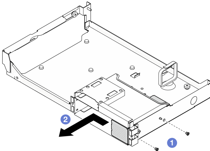
圖例 193. 卸下 E3.S 框架填充板
