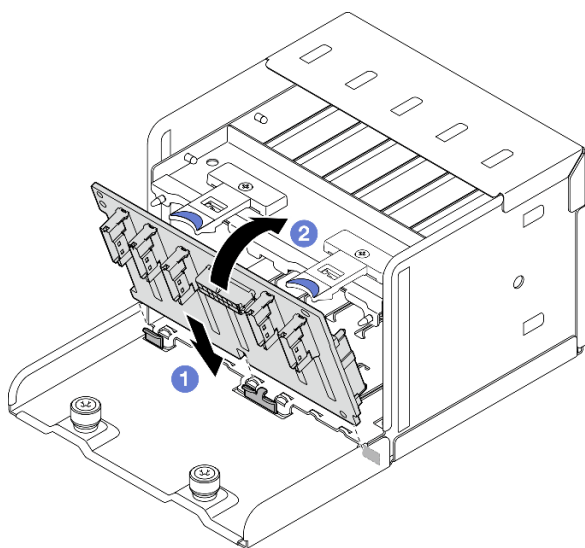
圖例 115. 2.5 吋硬碟背板安裝
