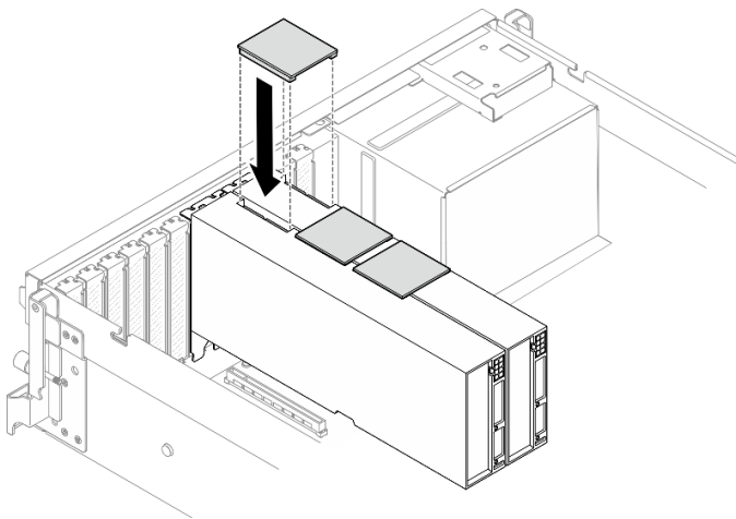
圖例 155. 安裝GPU 配接卡鏈結橋接器
