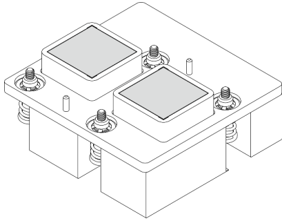
圖例 177. 擦掉 CX-7 散熱槽上的油灰墊
