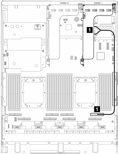
圖例 371. PCIe 擴充卡 1 纜線佈線
