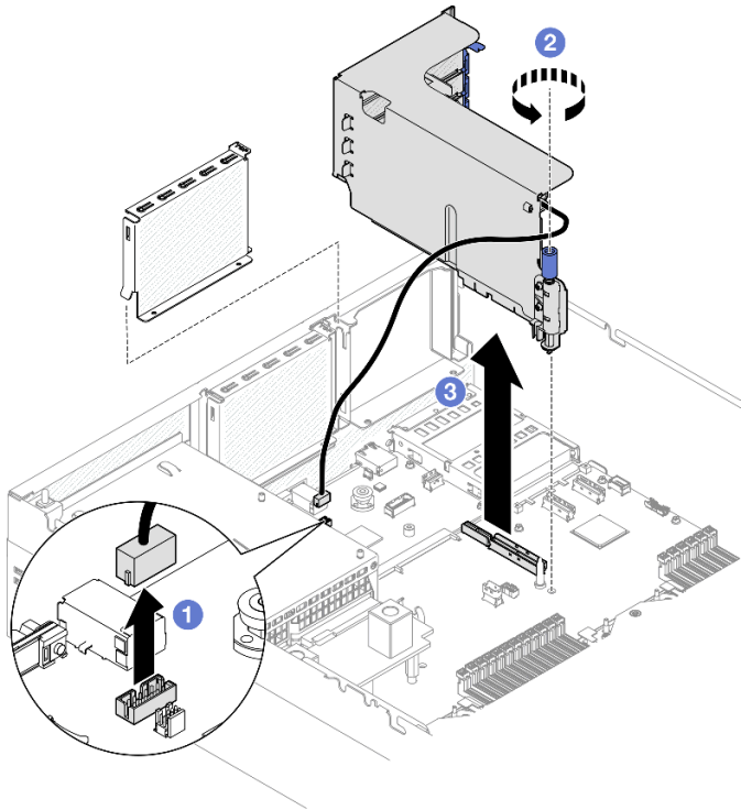
圖例 67. 卸下 PCIe 擴充卡 1 (含序列埠模組)
