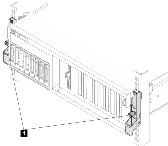
圖例 2. 使伺服器脫離機架
