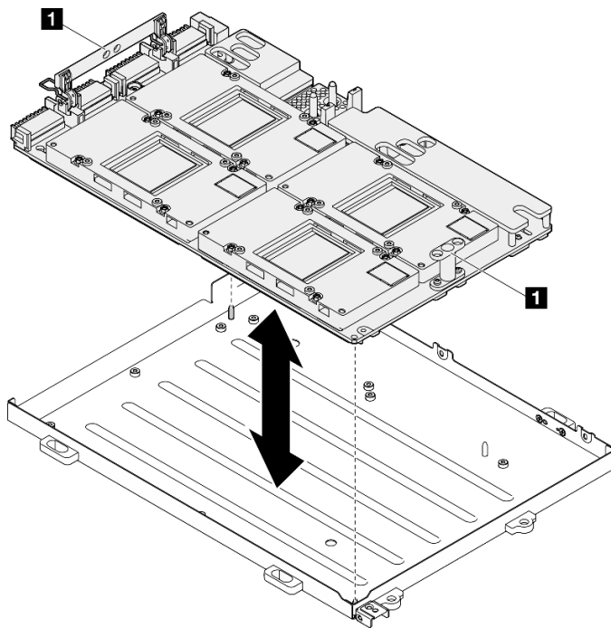
圖例 267. 安裝 SXM5 GPU 板組件
