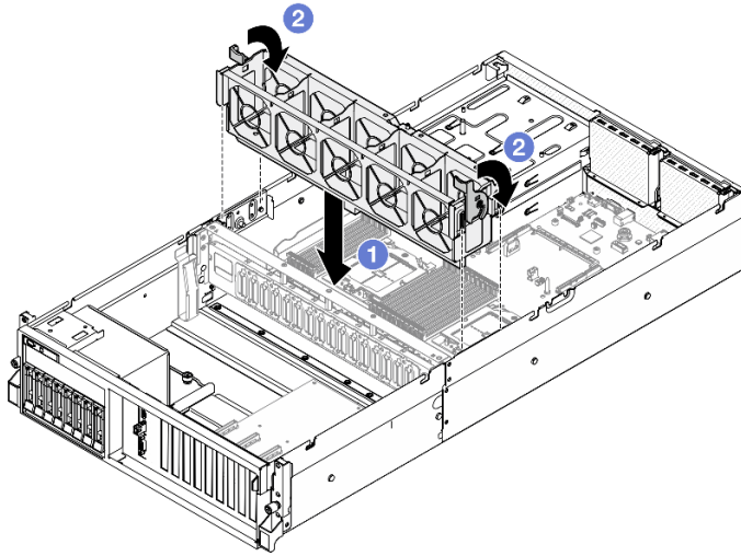
圖例 22. 安裝風扇機盒
