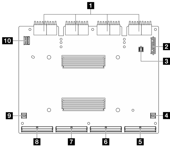
圖例 283. CX-7 支架板接頭
