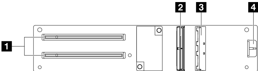
圖例 291. 正面 I/O 擴充板接頭
