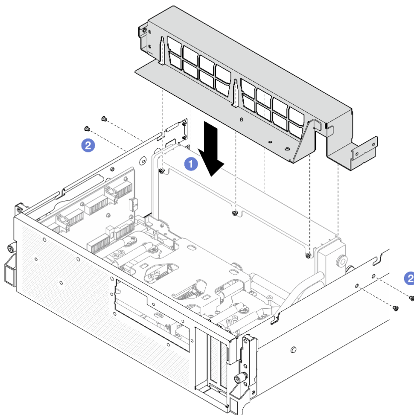
圖例 212. 安裝散熱器托架
