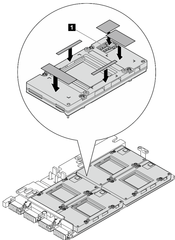
圖例 242. 貼附油灰墊
