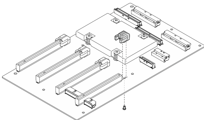
圖例 156. 卸下 PCIe 插槽加固件
