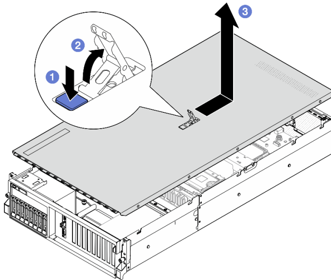
圖例 109. 卸下上蓋
