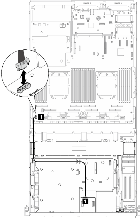
圖例 31. 拔除前方操作面板纜線 — SXM5 GPU 型號
