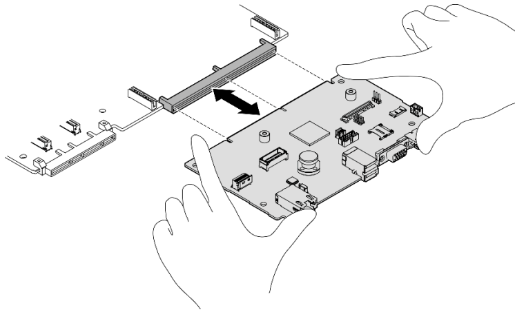
圖例 100. 安裝系統 I/O 板
