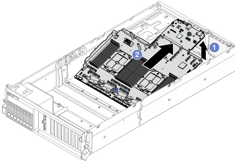
圖例 92. 卸下主機板組件
