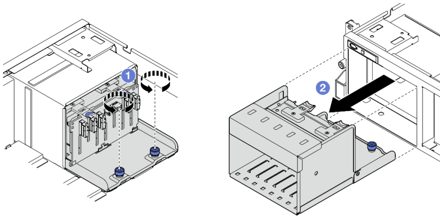
圖例 116. 卸下 2.5 吋框架組件
