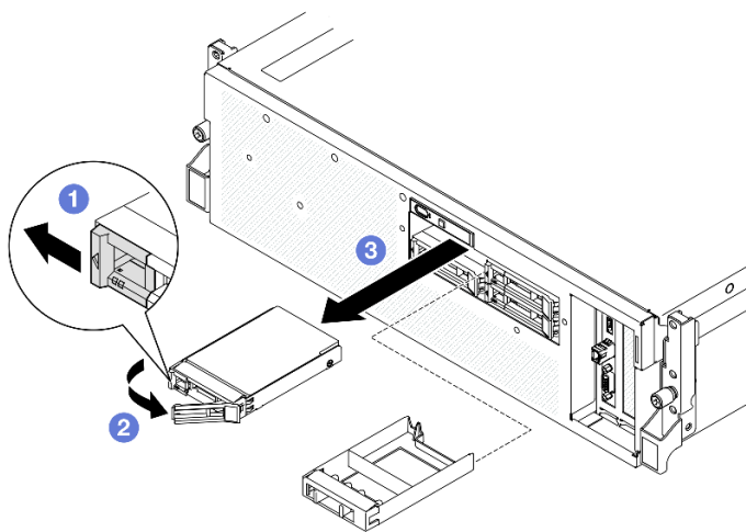
圖例 160. 卸下 2.5 吋熱抽換硬碟
