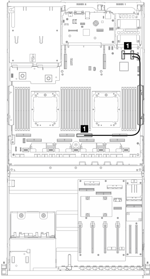
圖例 314. OCP 模組纜線佈線
