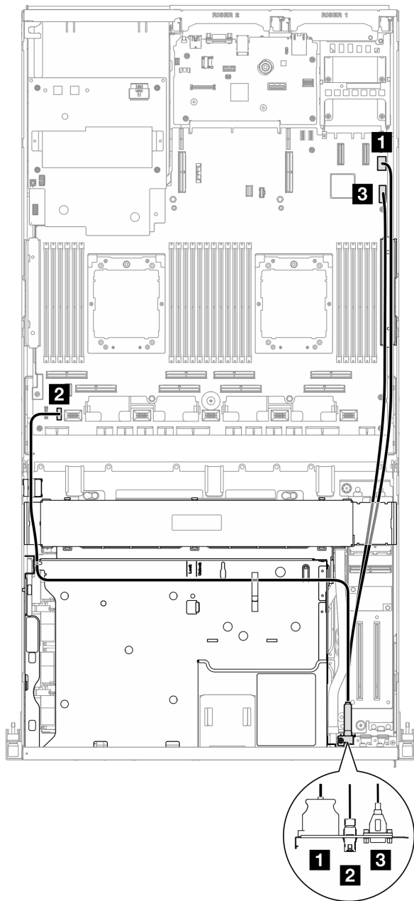
圖例 29. 正面 I/O 模組的纜線佈線 — SXM5 GPU 型號
