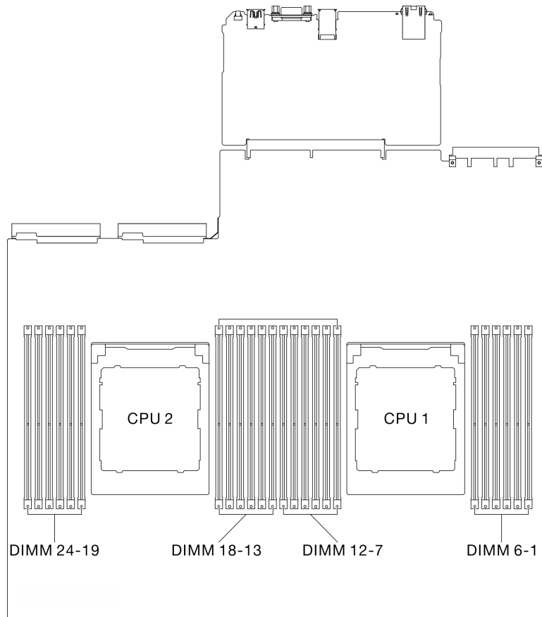
圖例 47. 記憶體模組和處理器佈置
