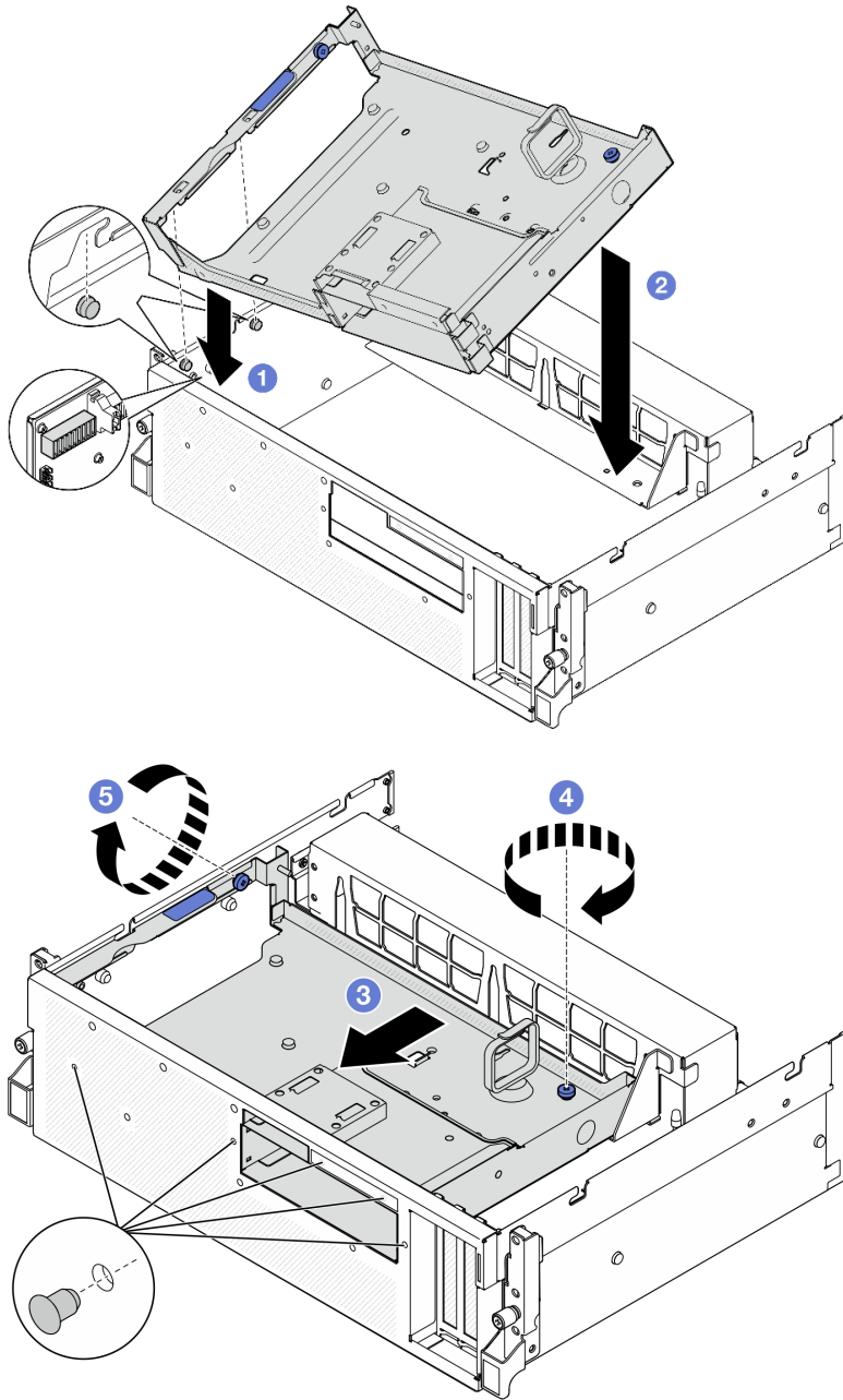
圖例 198. 安裝前方磁碟機托盤
