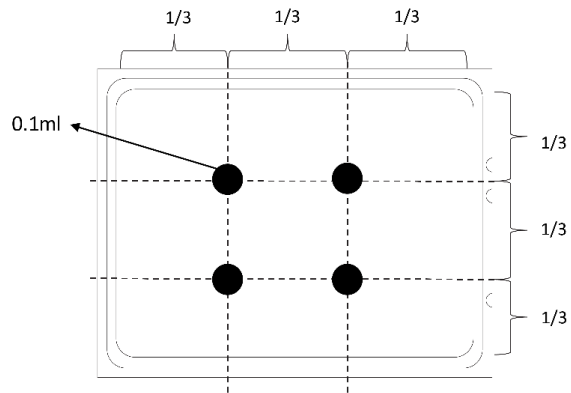
圖例 84. 塗上散熱膏
