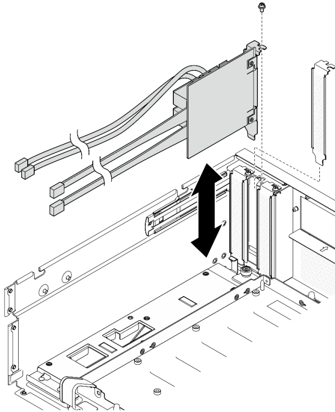
圖例 253. 安裝 OSFP 埠卡
