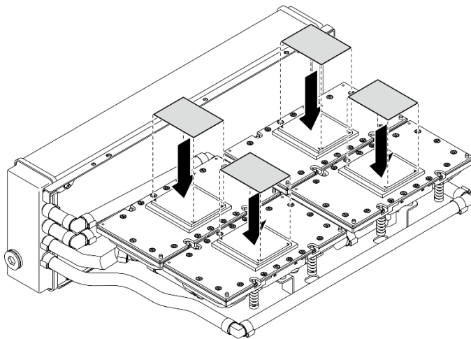
圖例 241. 貼附 PCM
