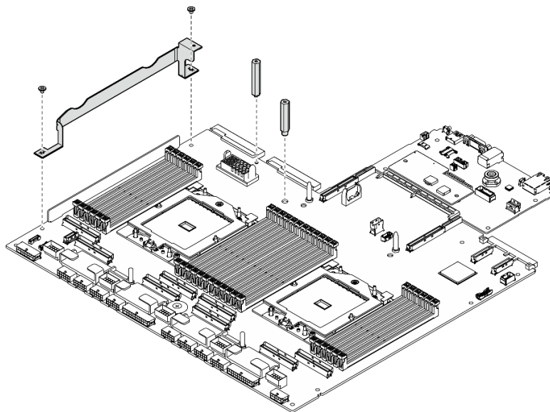
圖例 93. 卸下元件
