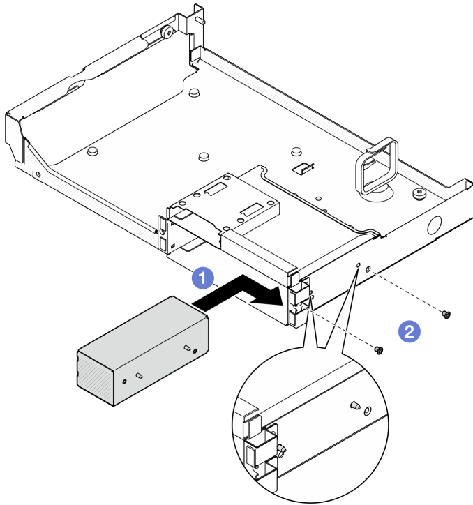
圖例 194. 安裝 E3.S 框架填充板
