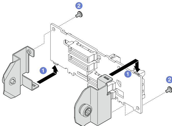
圖例 188. 安裝 E3.S 硬碟背板托架
