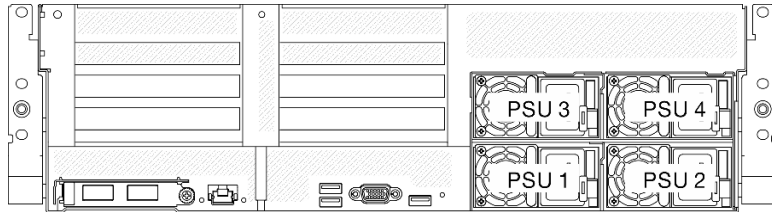
圖例 78. 電源供應器機槽編號
