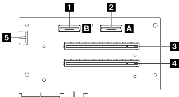
圖例 294. PCIe 擴充卡接頭
