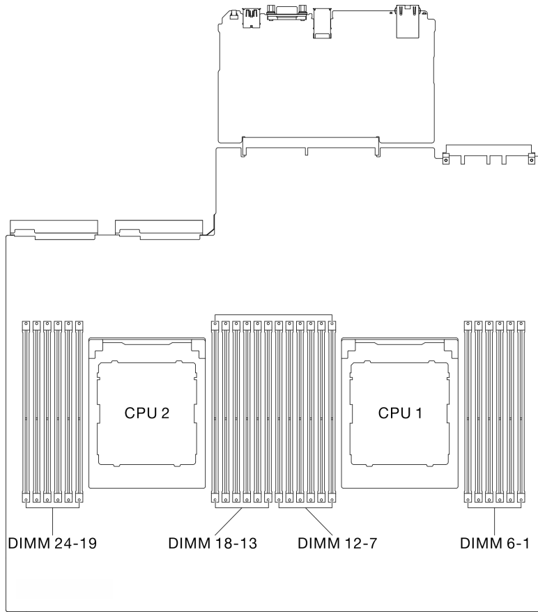
圖例 50. 記憶體模組和處理器佈置
