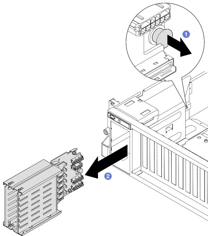
圖例 134. 卸下 E1.S 框架組件
