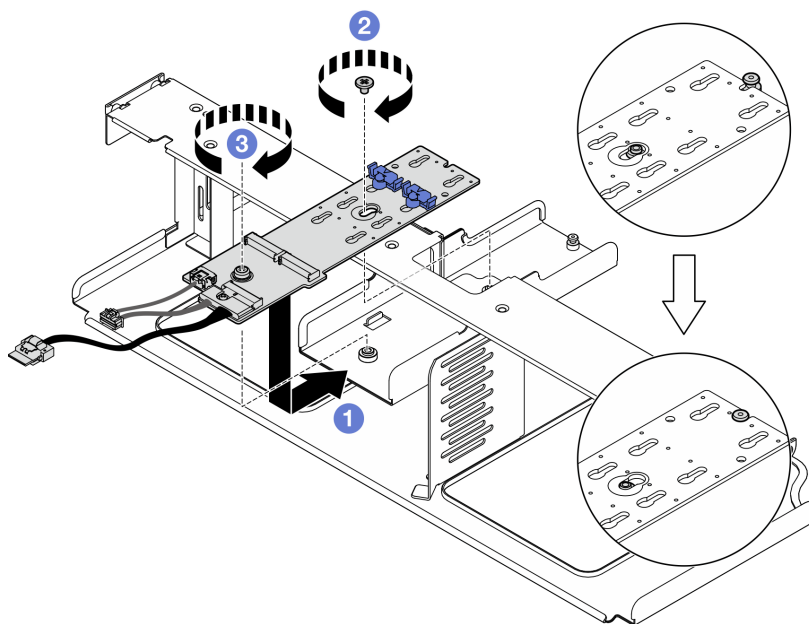
圖例 45. M.2 背板安裝
