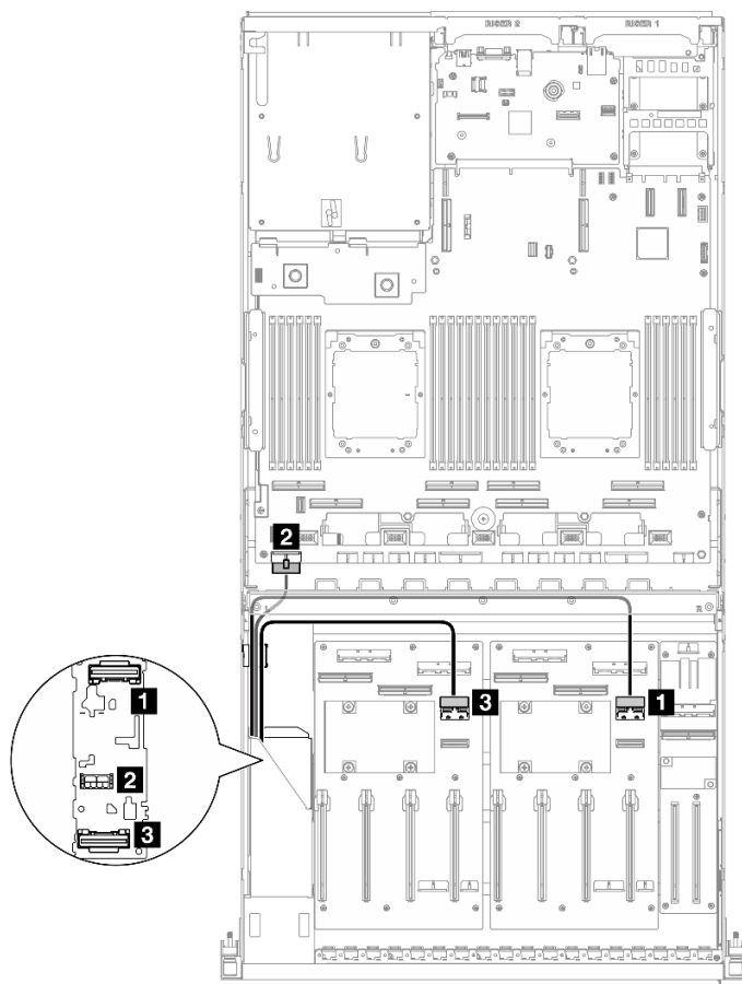
圖例 321. E3.S 硬碟背板纜線佈線
