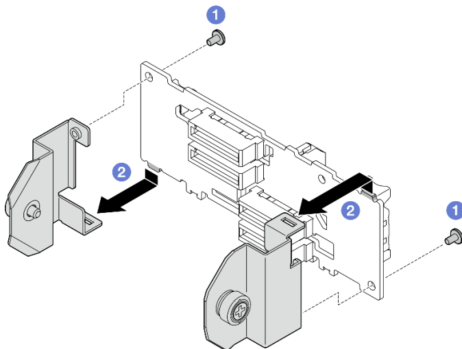
圖例 131. 卸下 E3.S 硬碟背板托架
