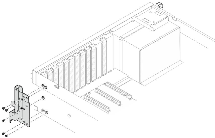
圖例 57. 安裝右安裝把手
