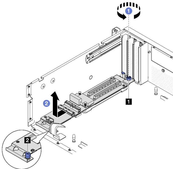
圖例 202. 卸下正面 I/O 擴充板模組
