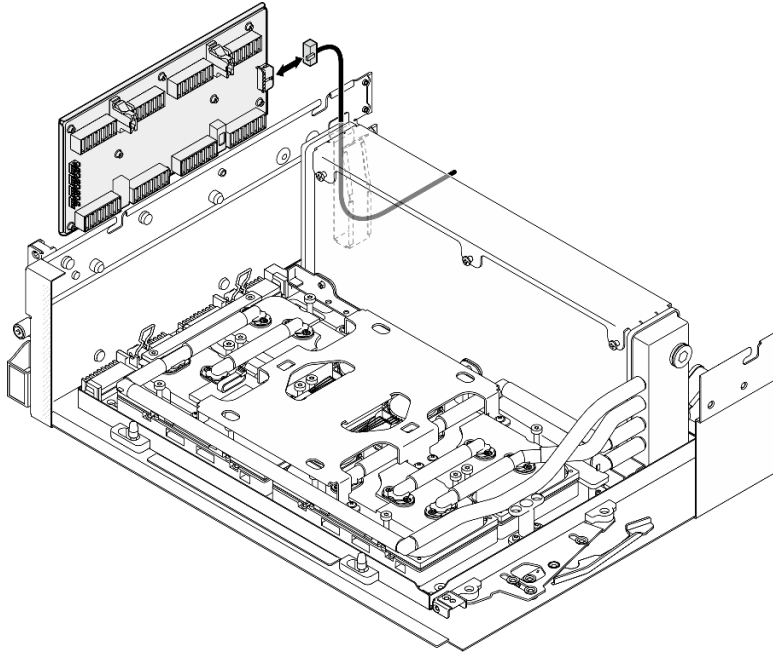
圖例 223. 轉插卡電源線連接
