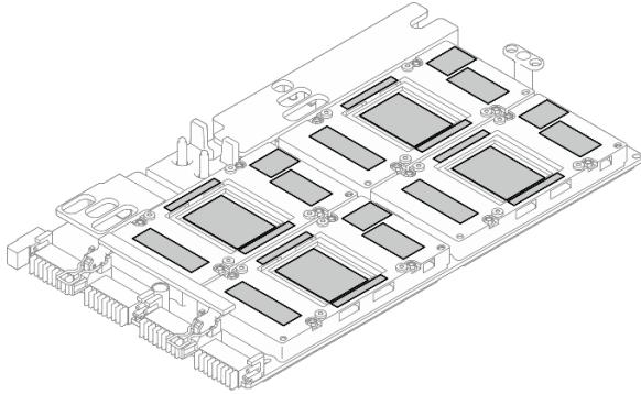
圖例 239. 擦掉 SXM5 GPU 上的 PCM 和油灰墊
