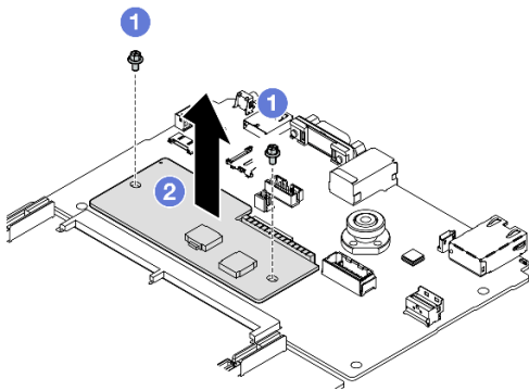
圖例 89. 卸下韌體和 RoT 安全模組
