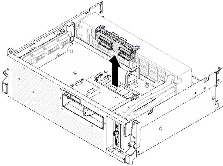
圖例 163. 卸下 2.5 吋硬碟背板模組
