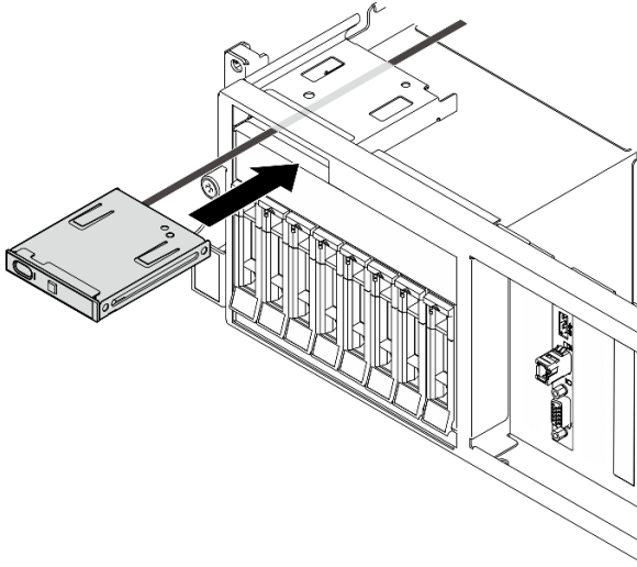
圖例 33. 安裝前方操作面板
