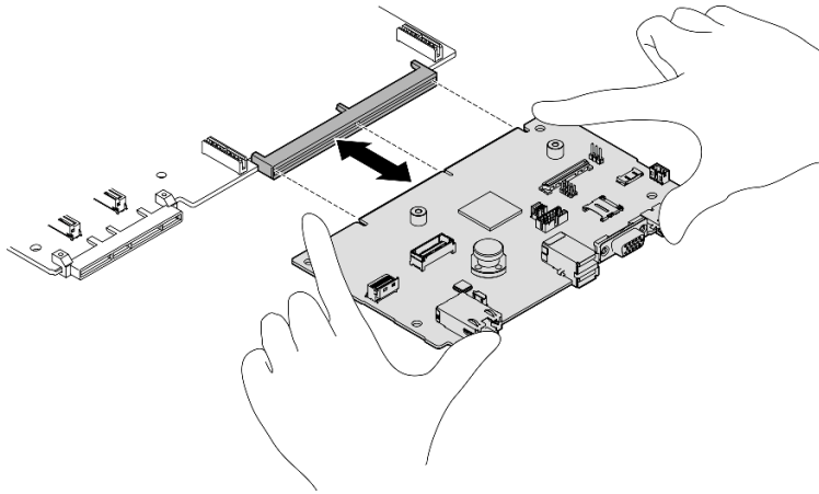
圖例 99. 卸下系統 I/O 板
