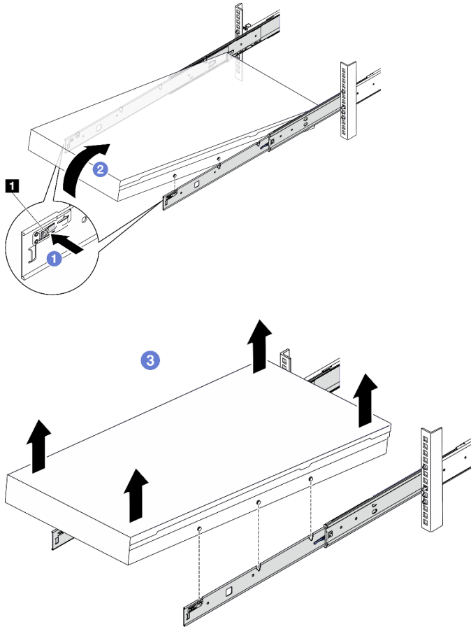
圖例 5. 從機架卸下伺服器
