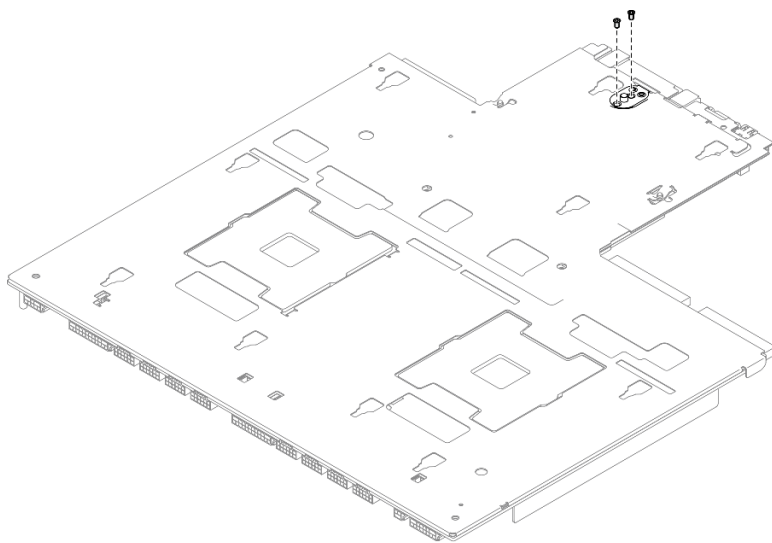
圖例 104. 安裝螺絲
