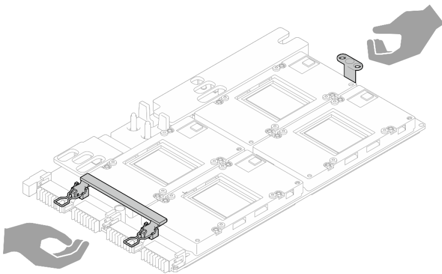
圖例 266. 從包裝盒取出 SXM5 GPU 板組件
