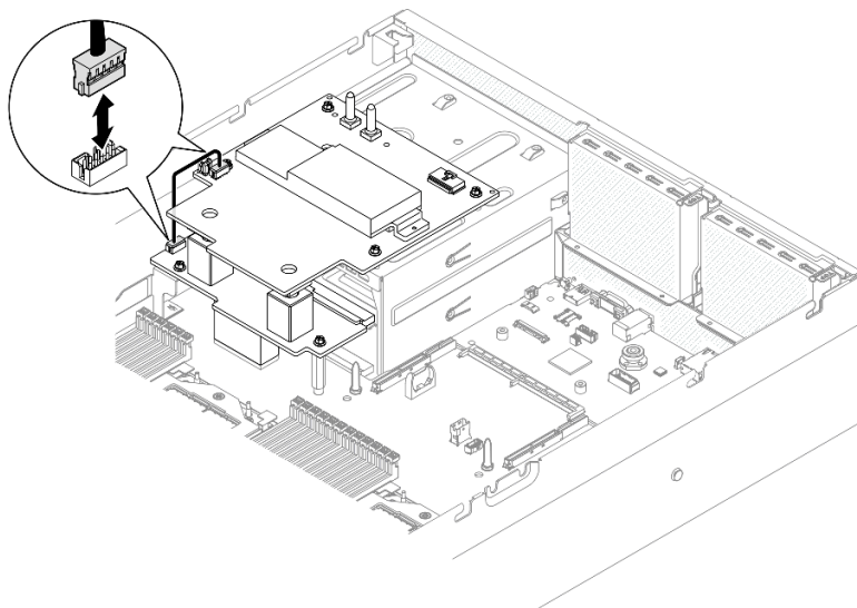
圖例 272. 拔掉側頻纜線
