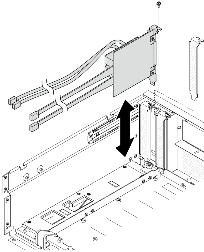
圖例 251. 卸下 OSFP 埠卡
