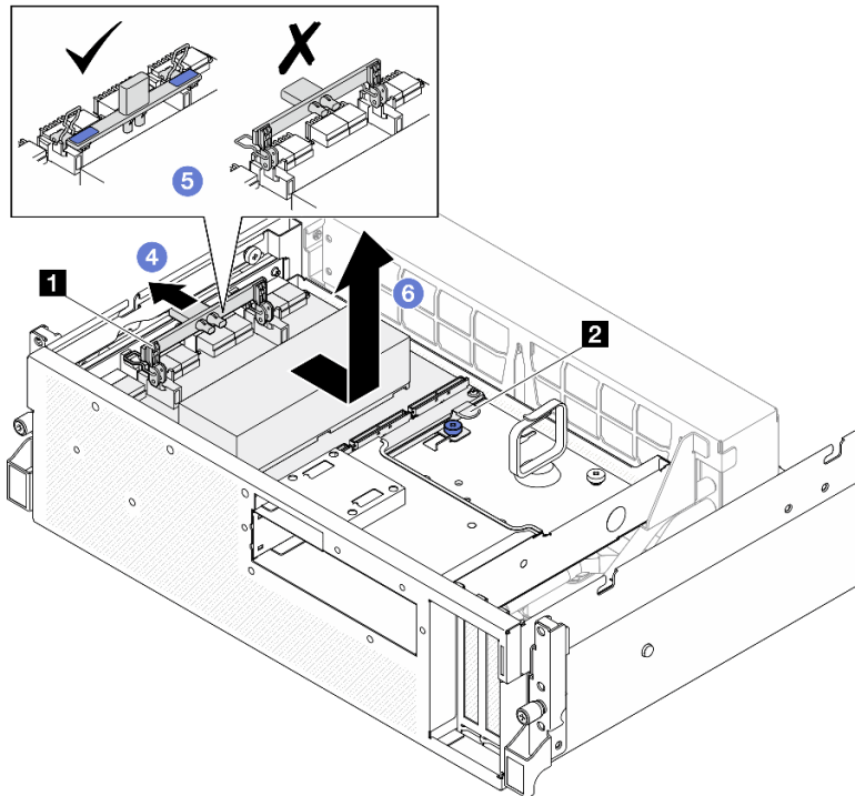
圖例 169. 卸下 CX-7 組件
