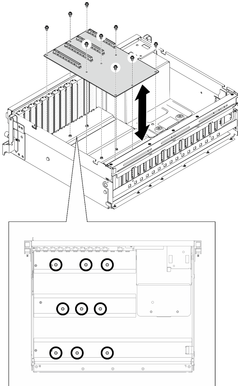
圖例 149. 安裝 GPU 配電板 — 4-DW GPU 型號
