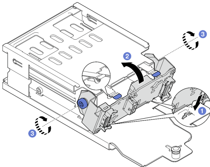
圖例 133. 安裝 E3.S 硬碟背板模組
