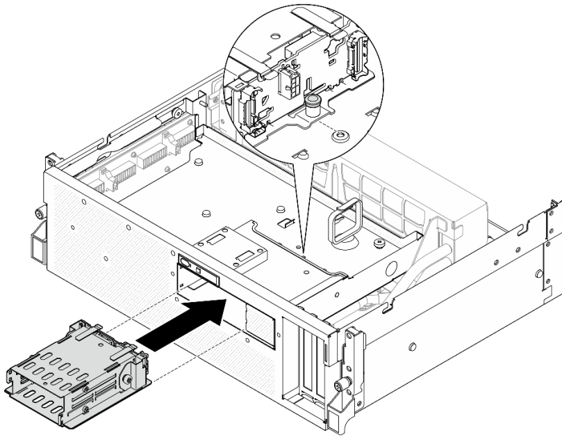
圖例 191. E3.S 框架組件安裝
