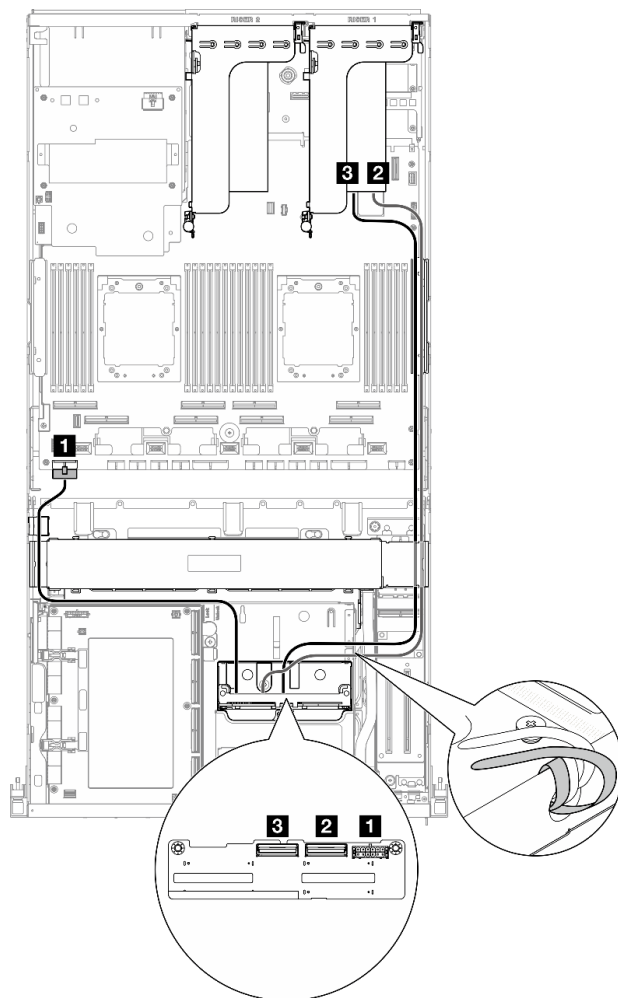
圖例 341. 2.5 吋硬碟背板纜線佈線 (RAID 配接卡在 PCIe 擴充卡 1 上)
