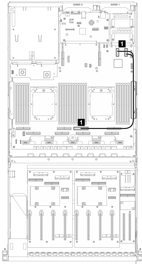
圖例 332. OCP 模組纜線佈線
