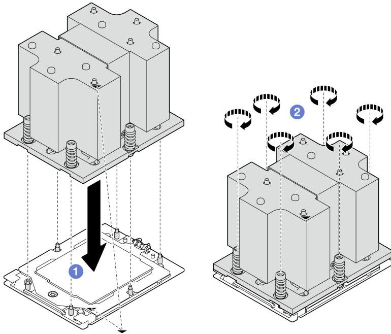
圖例 85. 安裝散熱槽
