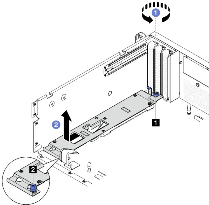
圖例 210. 卸下正面 I/O 擴充板支架
