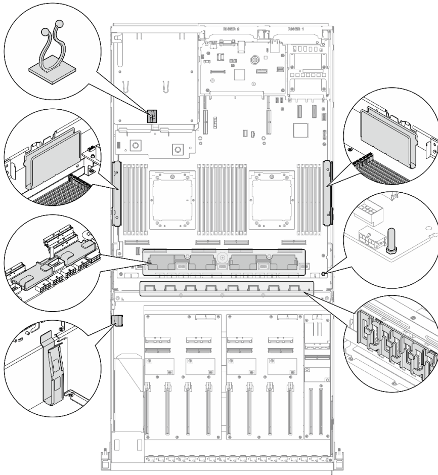
圖例 316. 機箱中的纜線導件和纜線夾位置
