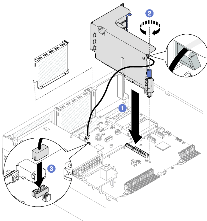
圖例 71. 安裝 PCIe 擴充卡 1 (含序列埠模組)
