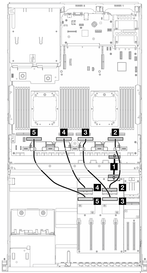
圖例 307. 直接 GPU 配電板纜線佈線
