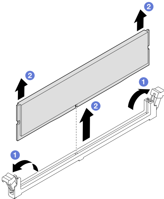
圖例 49. 卸下記憶體模組
