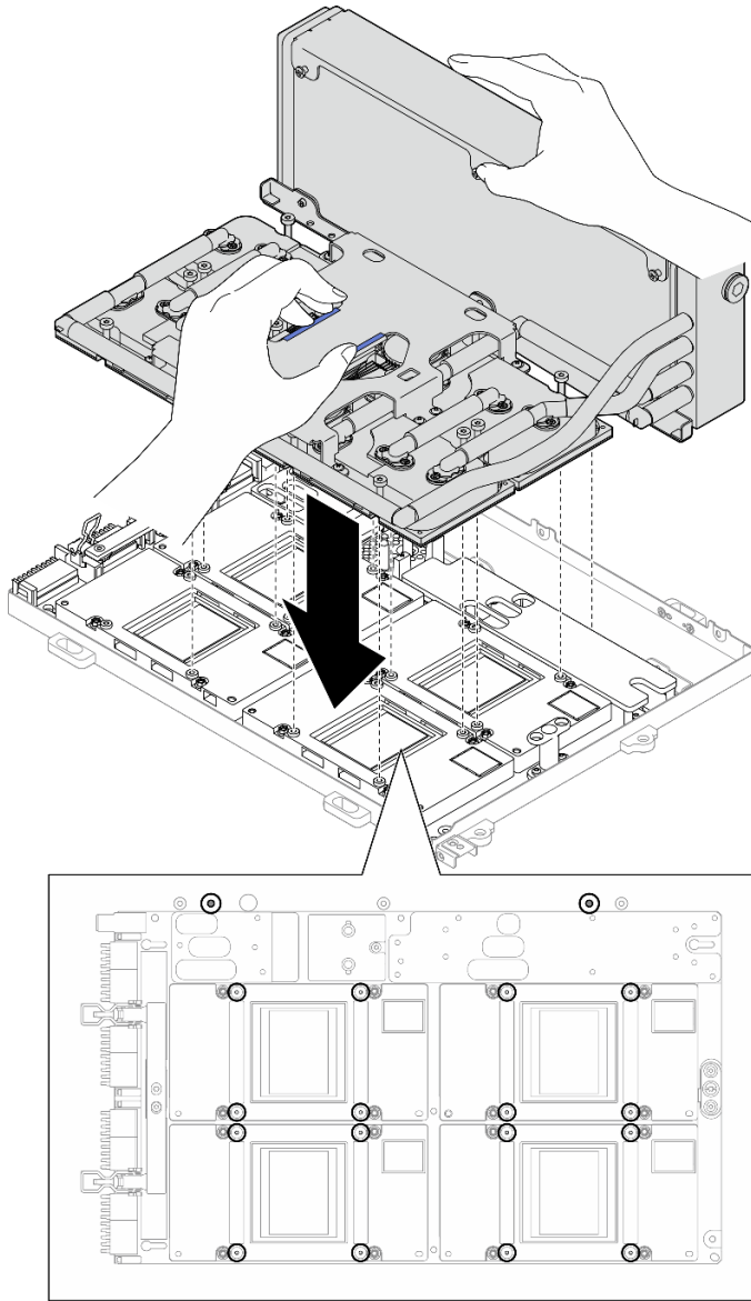
圖例 244. 安裝 L2A
