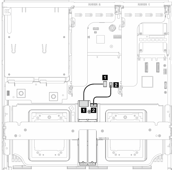
圖例 309. SATA/x4 NVMe M.2 背板纜線佈線
