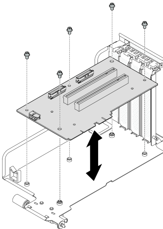
圖例 73. 卸下 PCIe 擴充卡
