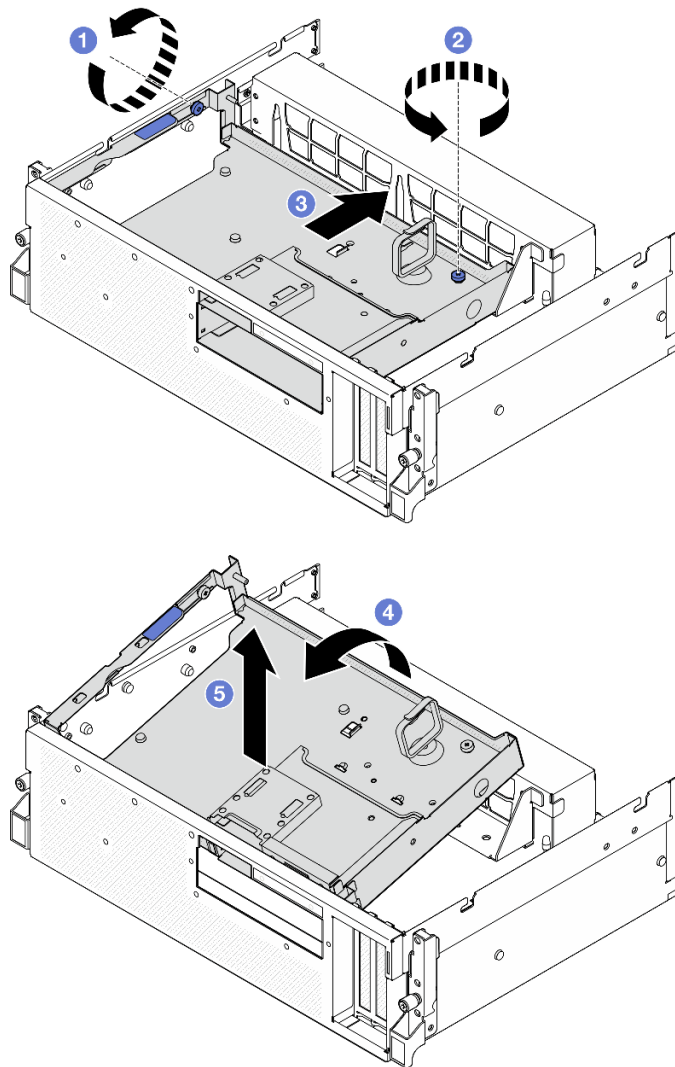
圖例 197. 卸下前方磁碟機托盤
