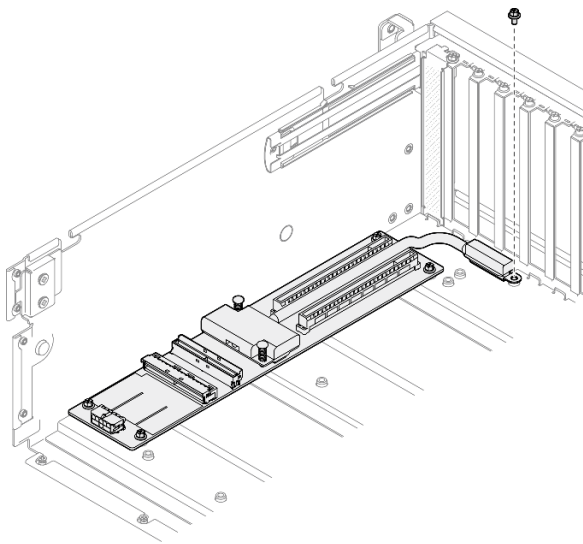
圖例 141. 安裝螺絲
