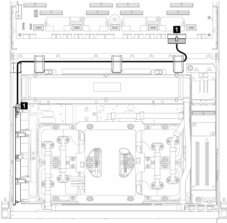
圖例 359. 轉插卡電源線佈線
