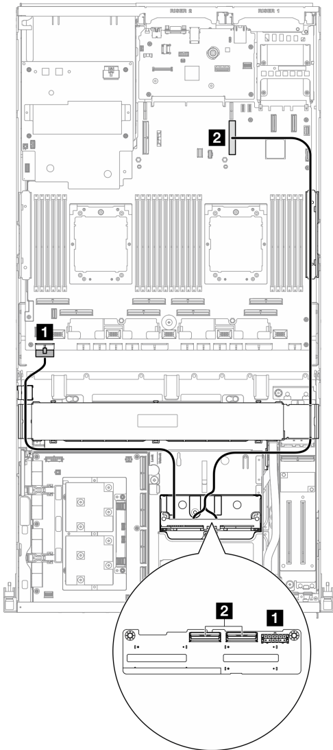
圖例 344. 2.5 吋硬碟背板纜線佈線
