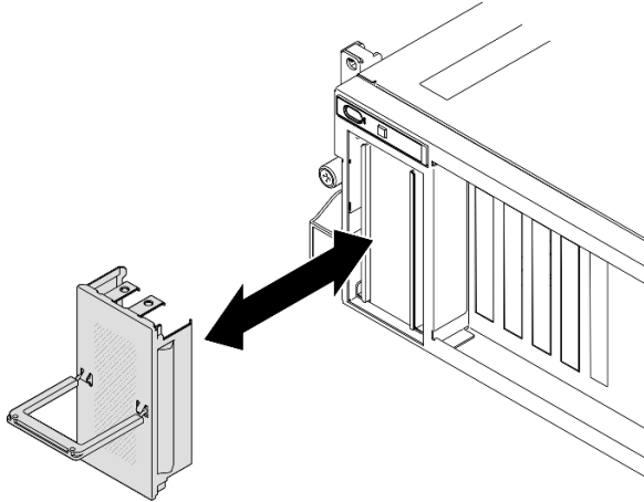
圖例 127. EDSFF 框架外蓋安裝
