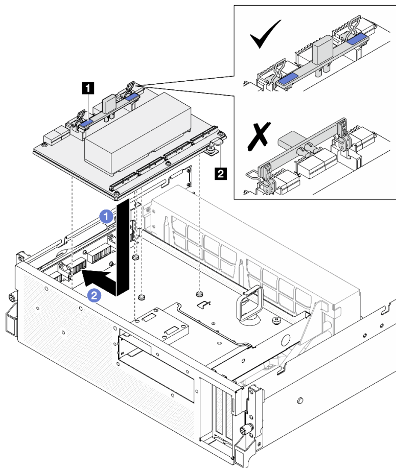
圖例 170. 安裝CX-7 組件
