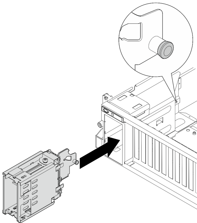
圖例 137. E3.S 框架組件安裝
