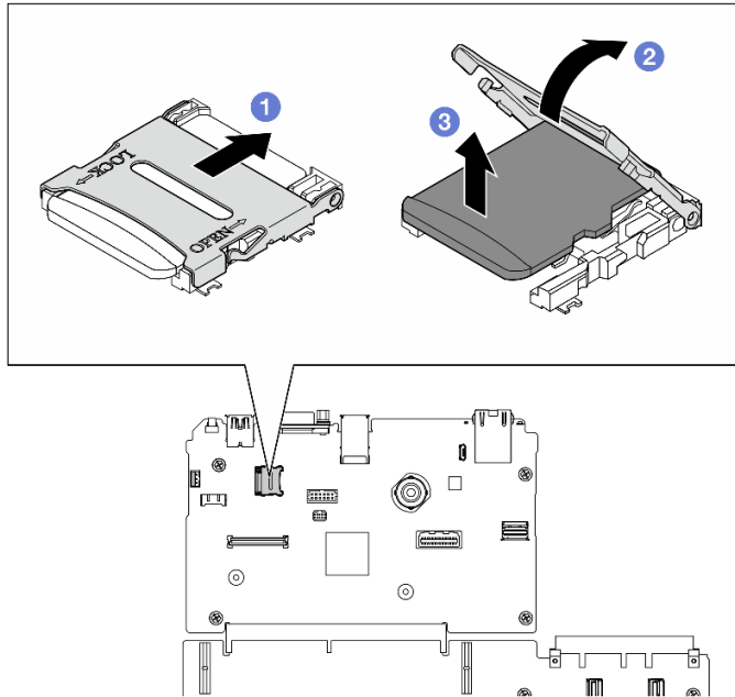
圖例 53. 卸下 MicroSD 卡
