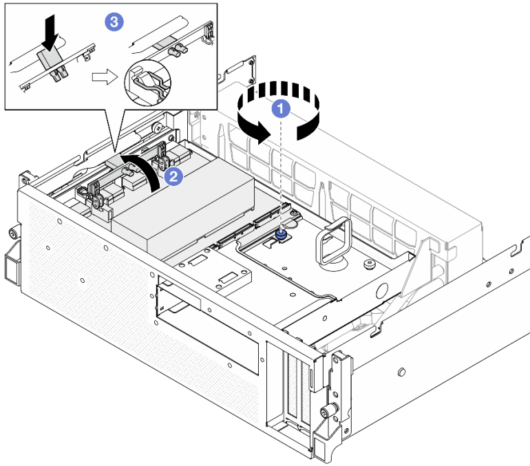
圖例 169. 卸下 CX-7 組件
