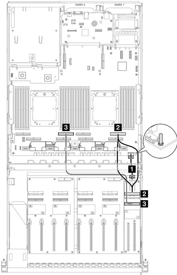
圖例 324. 正面 I/O 擴充板纜線佈線
