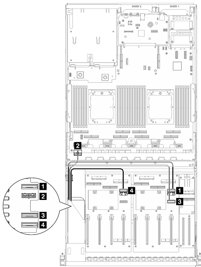
圖例 319. E1.S 硬碟背板纜線佈線
