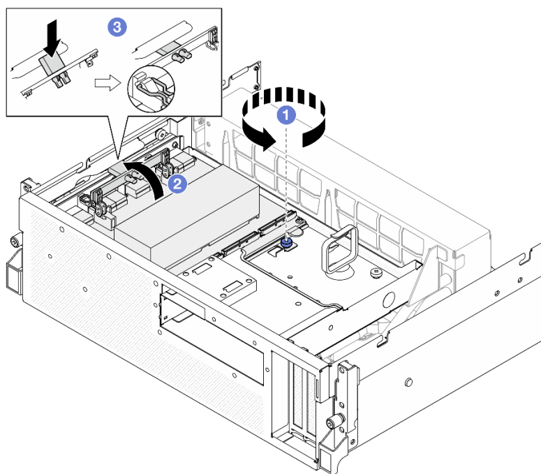
圖例 279. 卸下 SXM5 PCIe 交換器板
