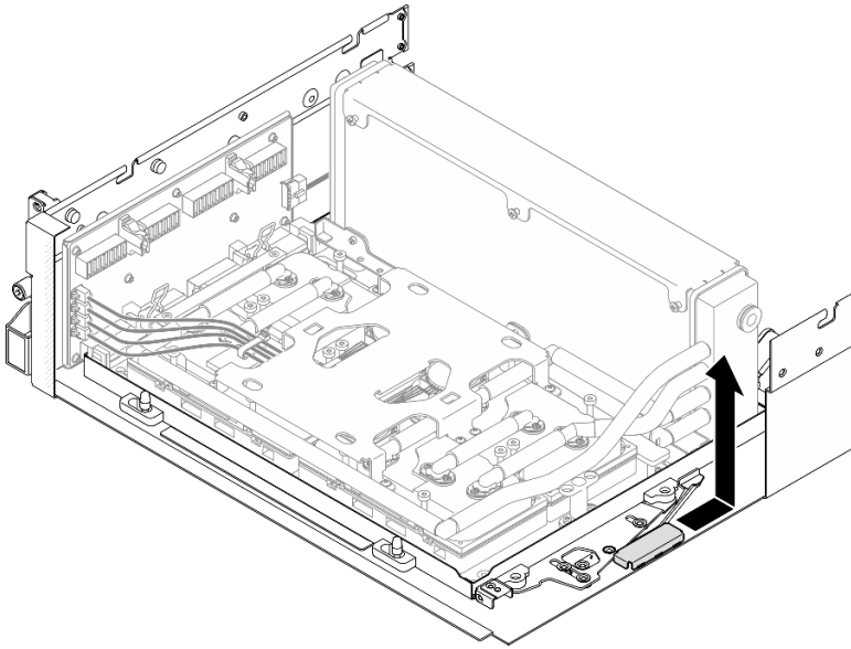
圖例 216. 卸下 SXM5 GPU 板組件固定托架
