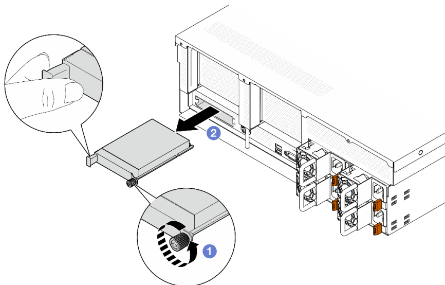
圖例 59. 卸下 OCP 模組
