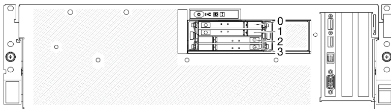
圖例 183. SXM5 GPU 型號中的 E3.S 熱抽換機槽編號
