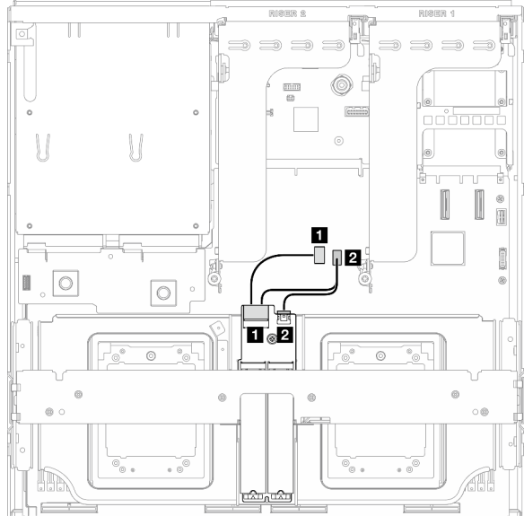
圖例 310. SATA/NVMe 或 NVMe RAID M.2 背板纜線佈線
