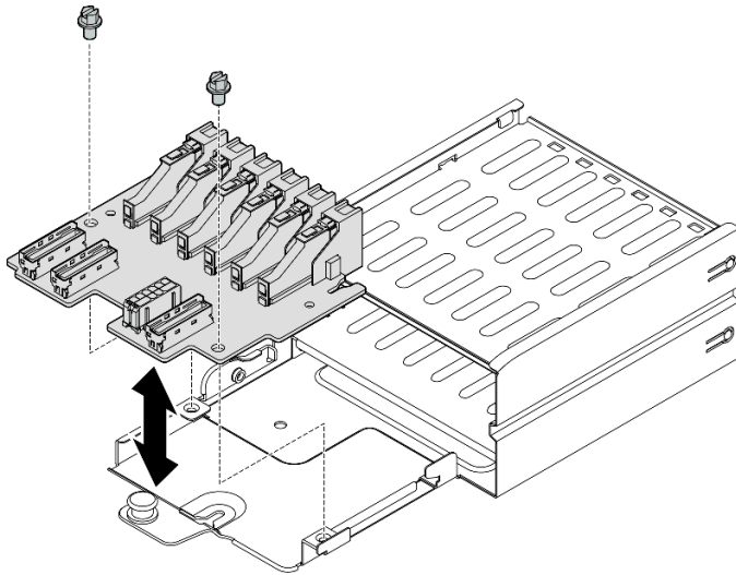
圖例 129. 安裝 E1.S 硬碟背板
