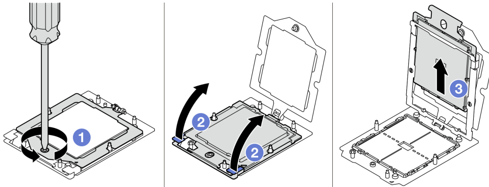
圖例 82. 卸下處理器
