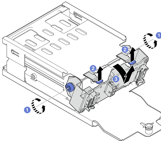
圖例 130. 卸下 E3.S 硬碟背板模組
