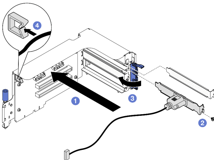
圖例 87. 序列埠模組安裝
