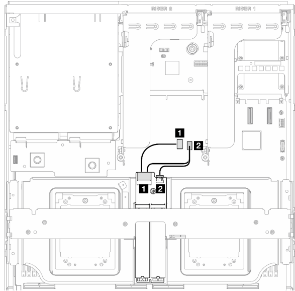
圖例 326. SATA/NVMe 或 NVMe RAID M.2 背板纜線佈線
