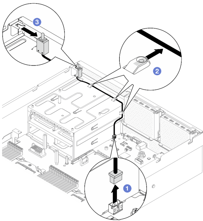
圖例 36. 卸下入侵開關
