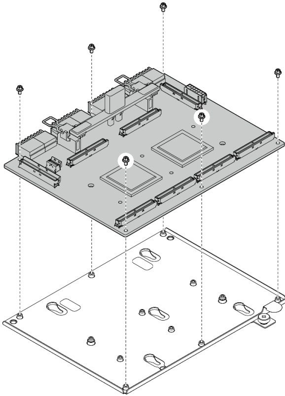
圖例 281. 拆卸 SXM5 PCIe 交換器板
