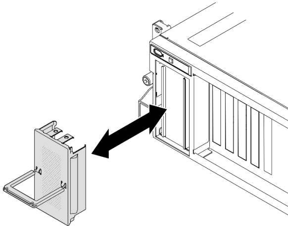
圖例 121. EDSFF 框架外蓋安裝
