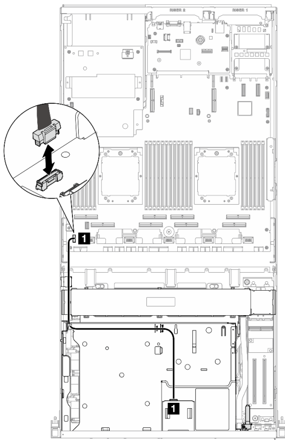
圖例 35. 前方操作面板的纜線佈線 — SXM5 GPU 型號
