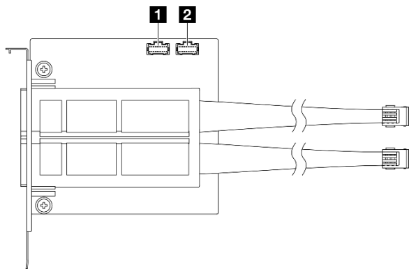
圖例 293. OSFP 埠卡 接頭
