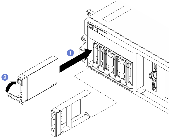
圖例 113. 安裝 2.5 吋熱抽換硬碟
