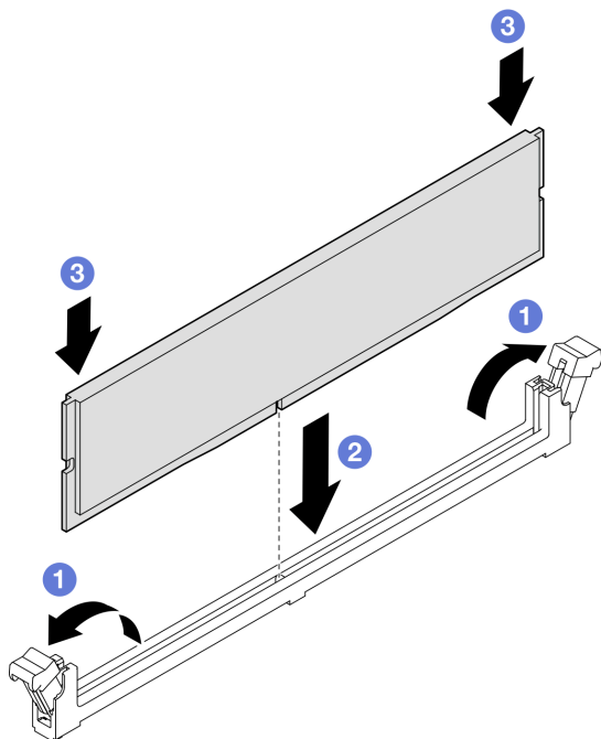
圖例 51. 安裝記憶體模組
