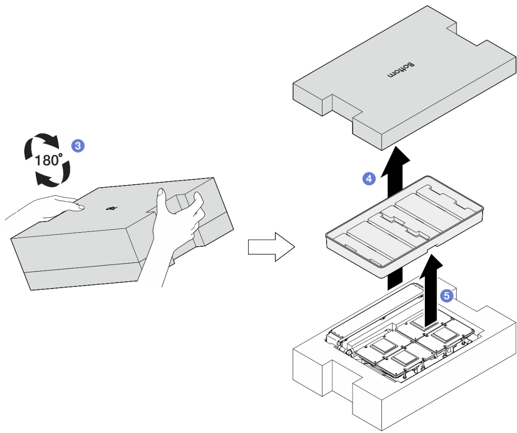
圖例 237. 將 L2A 上下倒置
