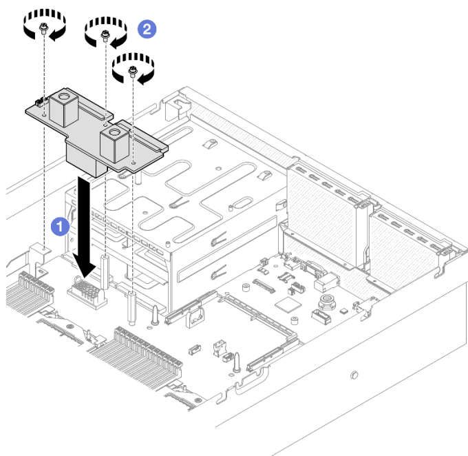
圖例 76. 安裝電源配送板
