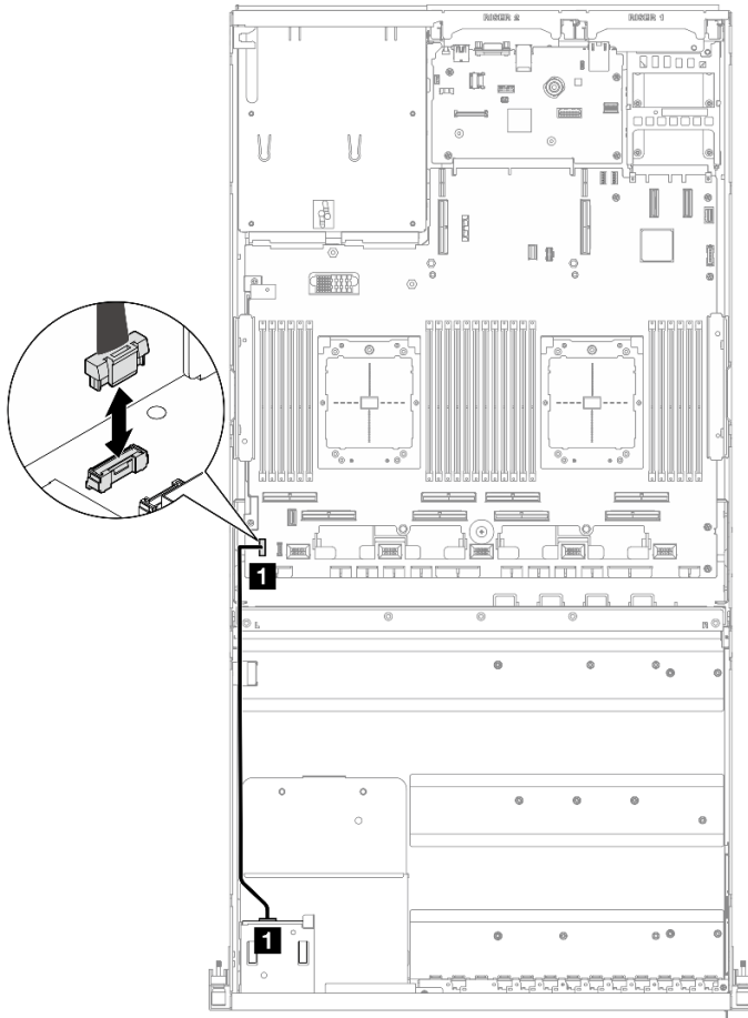
圖例 34. 前方操作面板的纜線佈線 — 4-DW GPU 型號和 8-DW GPU 型號
