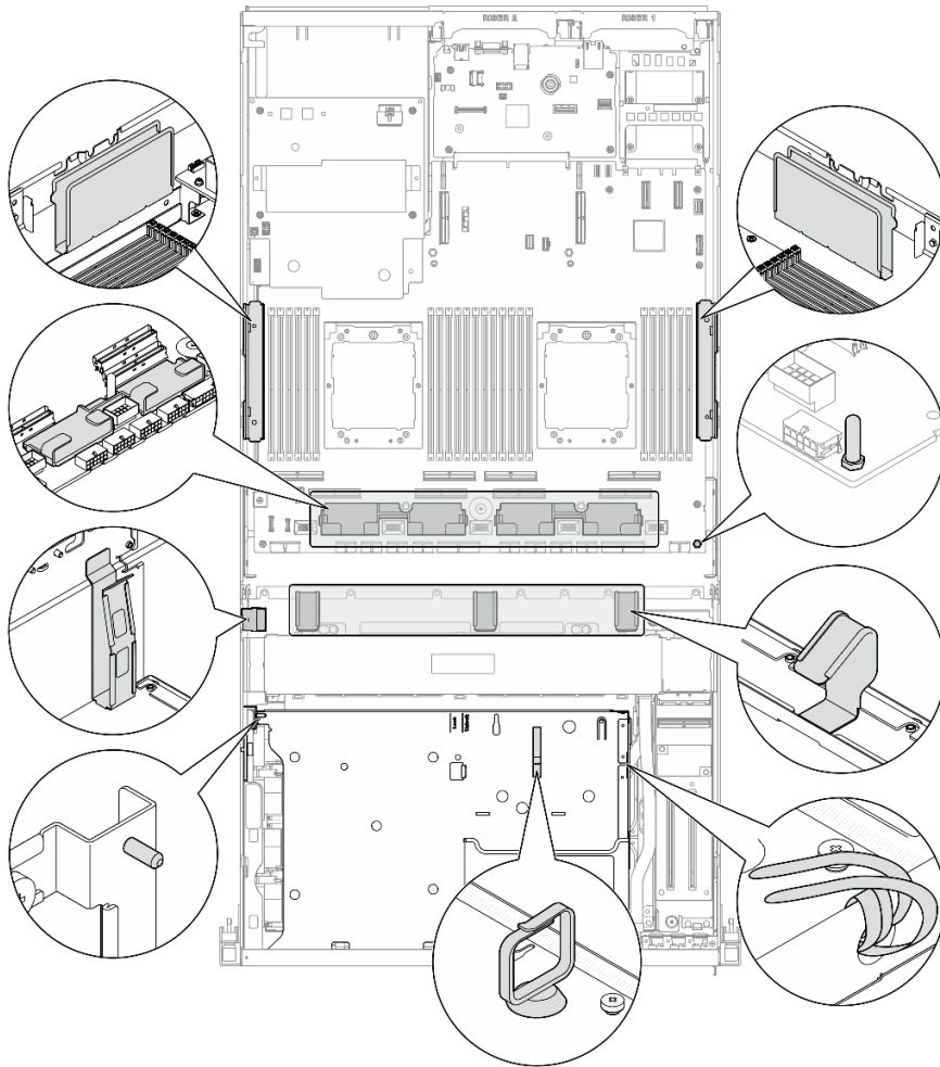
圖例 337. 機箱中的纜線導件、纜線夾、纜線固定導件和纜線束帶位置
