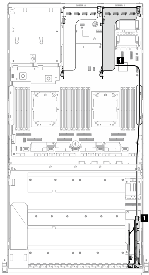
圖例 317. DPU 配接卡電源線佈線
