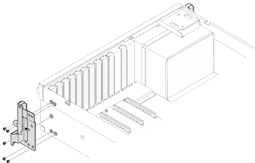
圖例 55. 卸下右安裝把手
