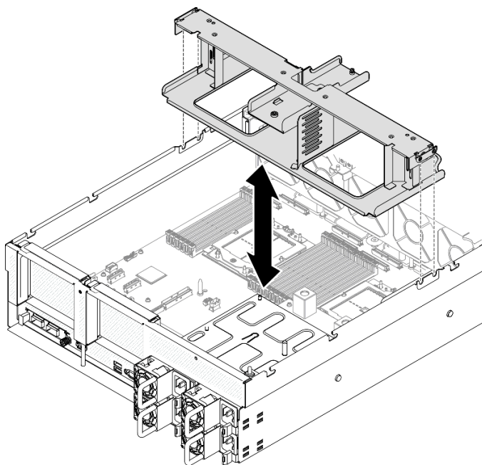
圖例 12. 卸下空氣擋板
