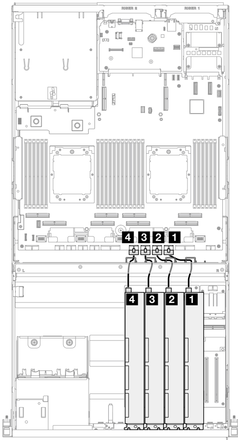
圖例 306. GPU 配接卡電源線佈線
