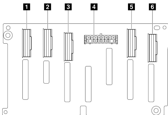
圖例 286. 8x 2.5 吋 SAS/SATA/NVMe 背板接頭
