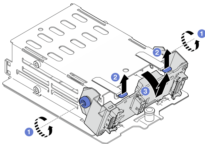
圖例 186. 卸下 E3.S 硬碟背板模組
