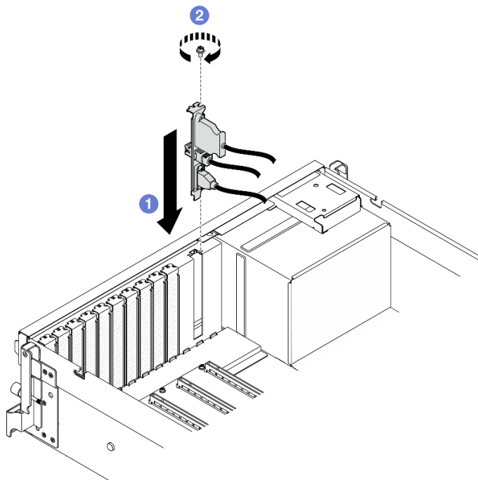
圖例 27. 安裝正面 I/O 模組
