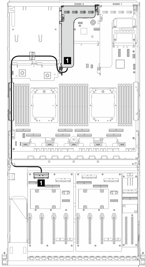
圖例 336. PCIe 擴充卡 2 纜線佈線
