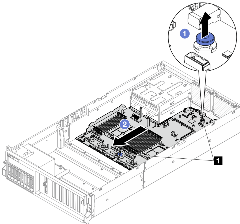
圖例 91. 鬆開主機板組件
