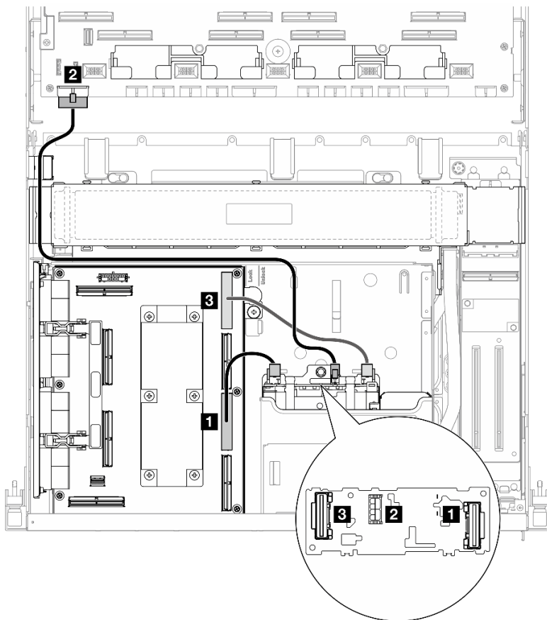
圖例 351. E3.S 硬碟背板纜線佈線
