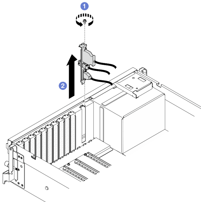
圖例 26. 卸下正面 I/O 模組
