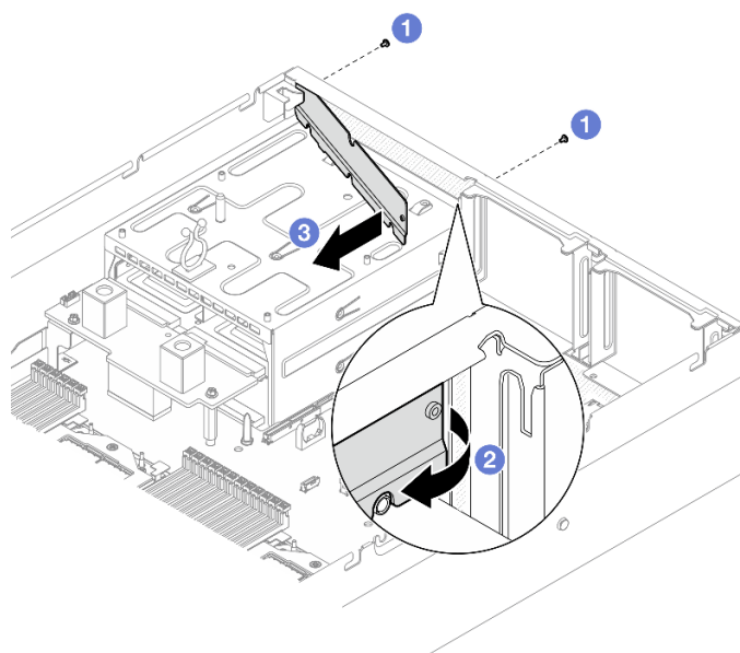
圖例 158. 卸下熱氣流後擋板
