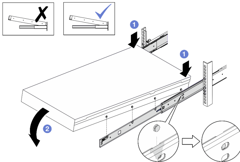
圖例 8. 將伺服器安裝到滑軌
