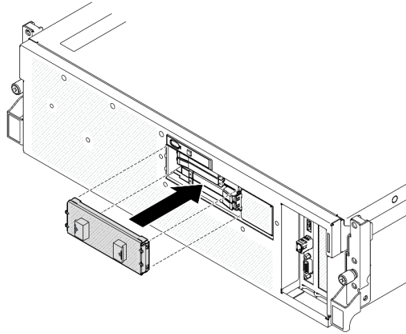
圖例 182. 安裝 E3.S 框架外蓋
