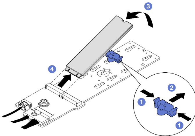
圖例 39. 卸下 M.2 硬碟
