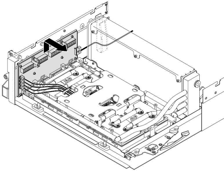
圖例 218. 鬆開轉插卡
