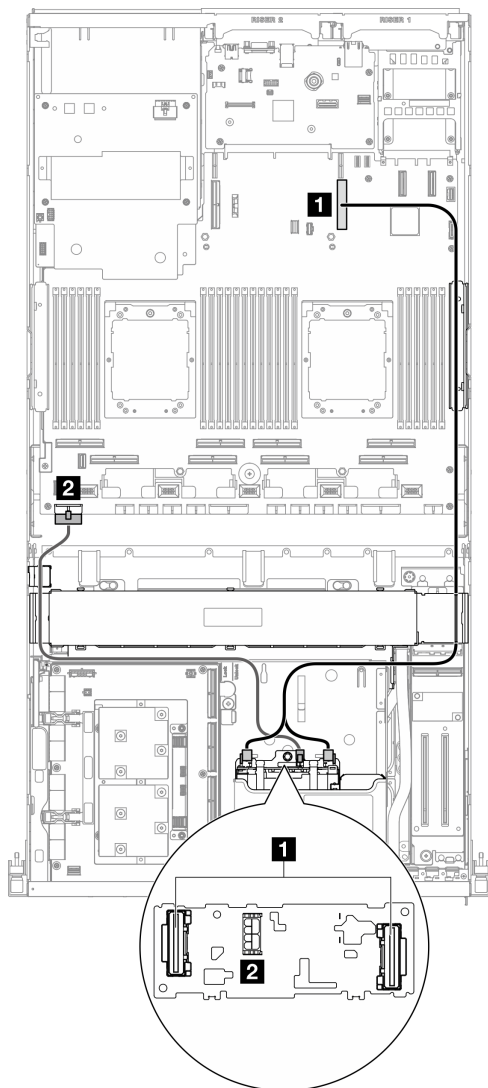
圖例 354. E3.S 硬碟背板纜線佈線
