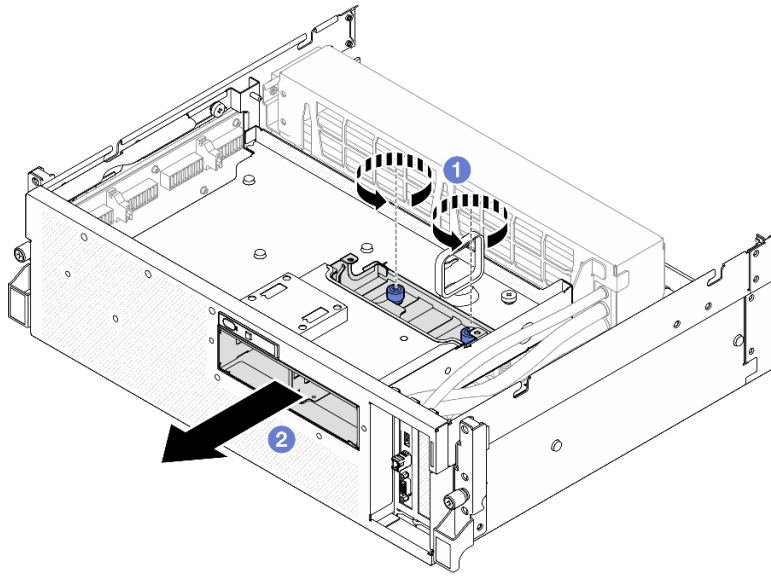
圖例 166. 卸下 2.5 吋框架
