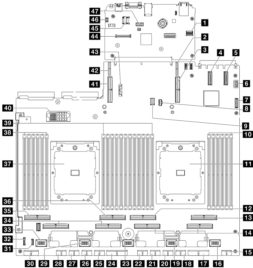
圖例 297. 主機板組件接頭
