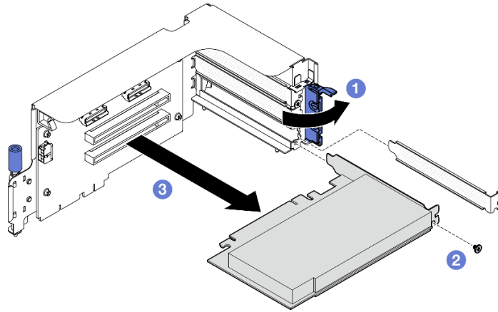
圖例 62. 卸下背面 PCIe 配接卡
