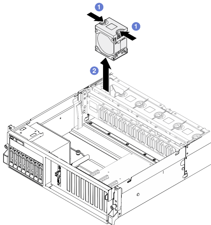
圖例 19. 卸下風扇
