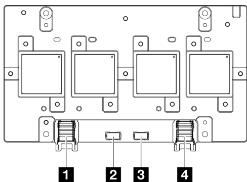
圖例 284. CX-7 Mezz 板接頭
