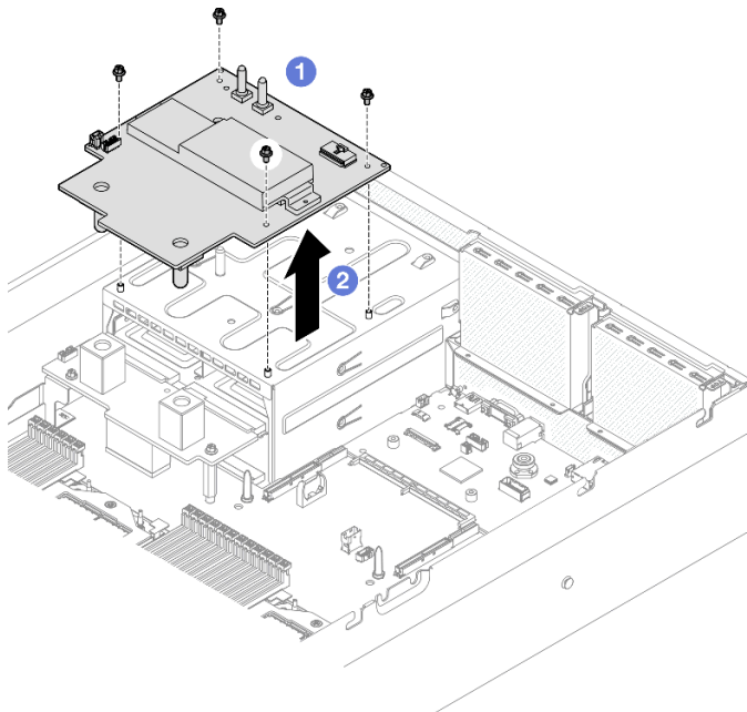
圖例 274. 卸下 SXM5 GPU 電源配送板
