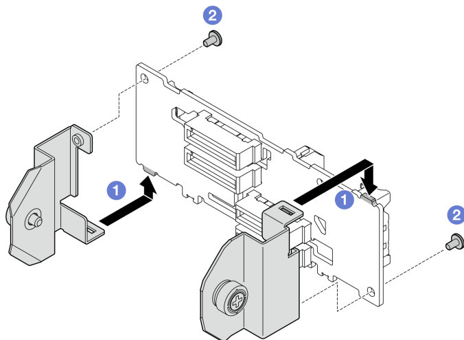
圖例 132. 安裝 E3.S 硬碟背板托架
