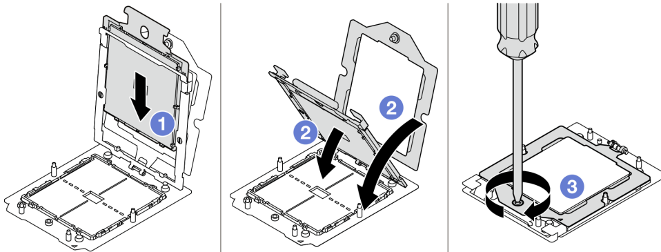
圖例 83. 安裝處理器
