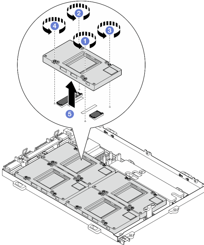
圖例 257. 卸下 SXM5 GPU
