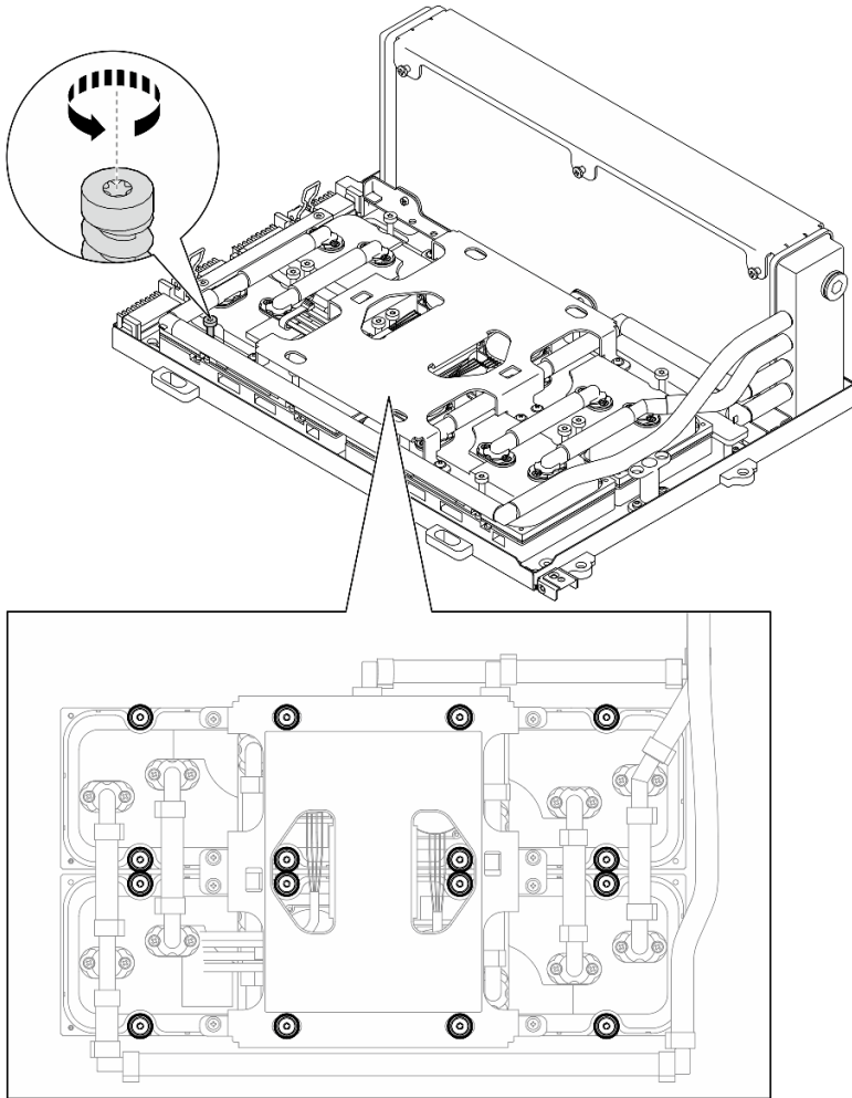
圖例 234. 卸下 Torx T15 螺絲
