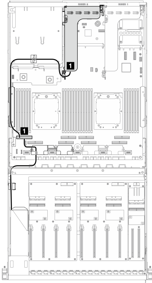
圖例 334. PCIe 擴充卡 2 纜線佈線
