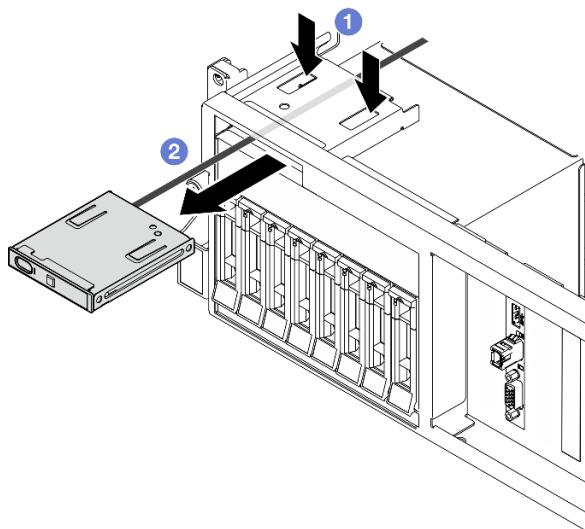
圖例 32. 卸下前方操作面板
