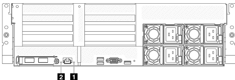
圖例 384. 背面圖上的系統 LED
