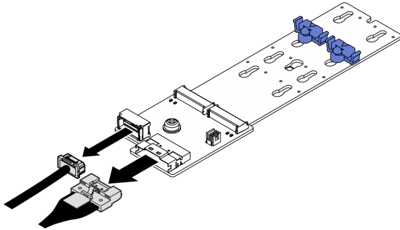
圖例 42. 拔除 SATA/x4 NVMe M.2 背板纜線
