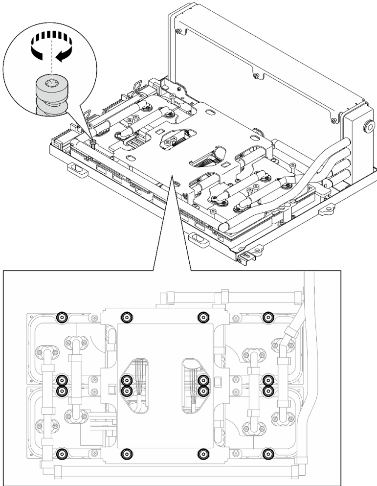
圖例 246. 安裝 Torx T15 螺絲
