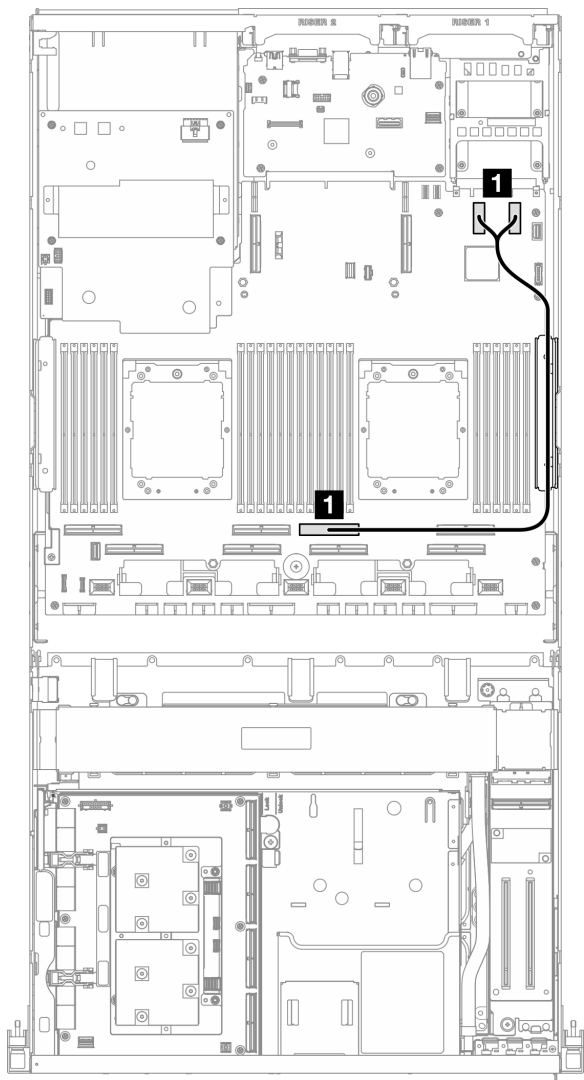
圖例 368. OCP 模組纜線佈線
