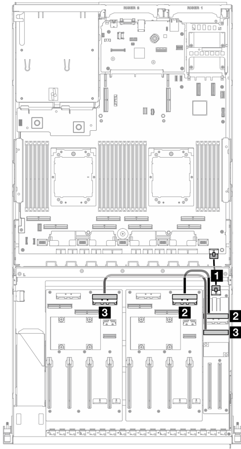
圖例 323. 正面 I/O 擴充板纜線佈線
