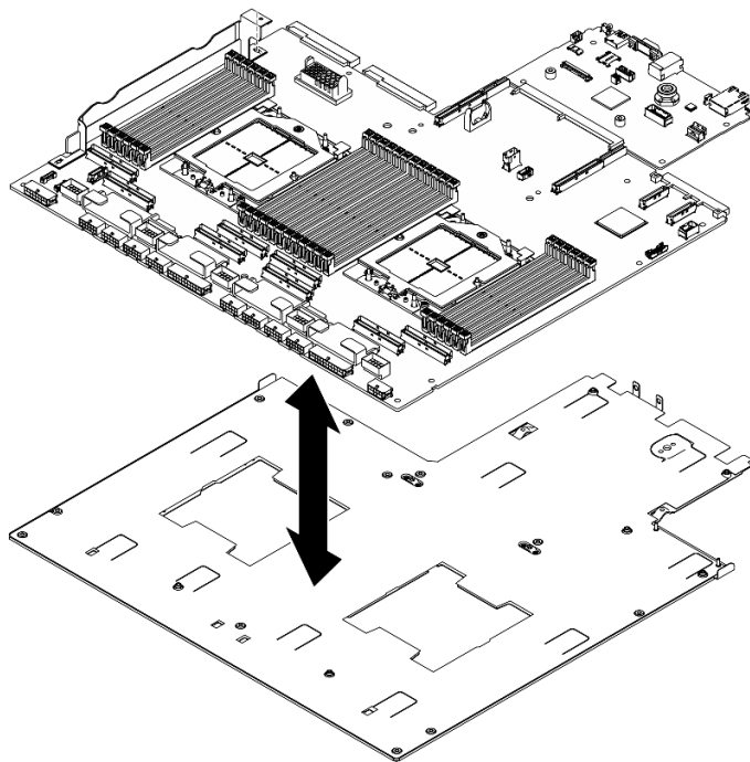
圖例 98. 拆卸主機板組件
