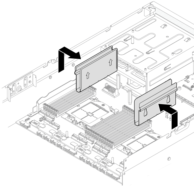
圖例 48. 卸下纜線導件
