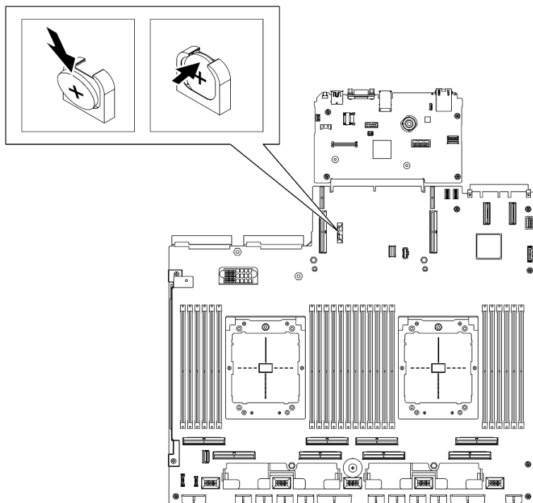
圖例 15. CMOS 電池安裝
