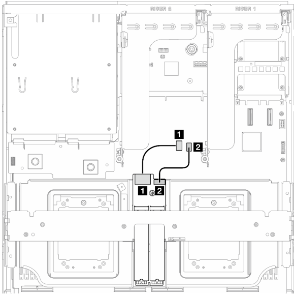
圖例 325. SATA/x4 NVMe M.2 背板纜線佈線
