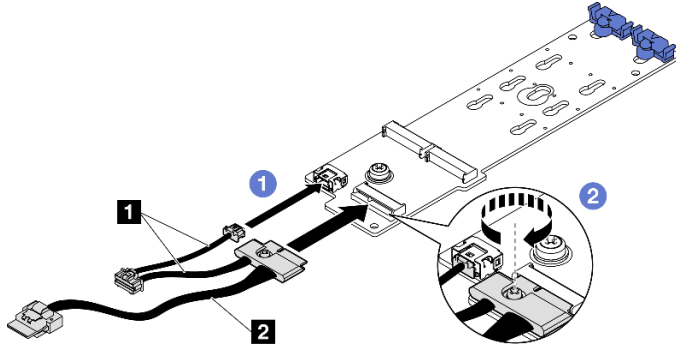
圖例 43. SATA/NVMe 或 NVMe RAID M.2 背板纜線連接
