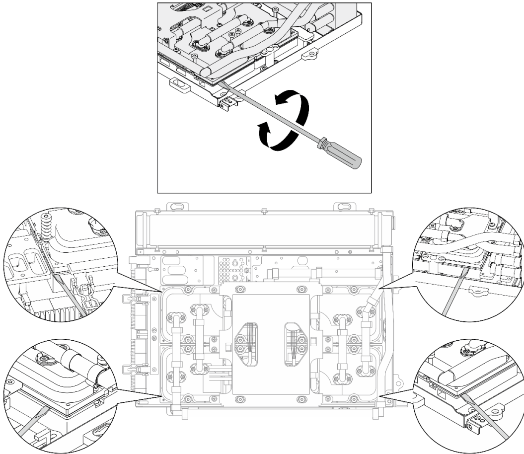
圖例 235. 鬆開水冷板
