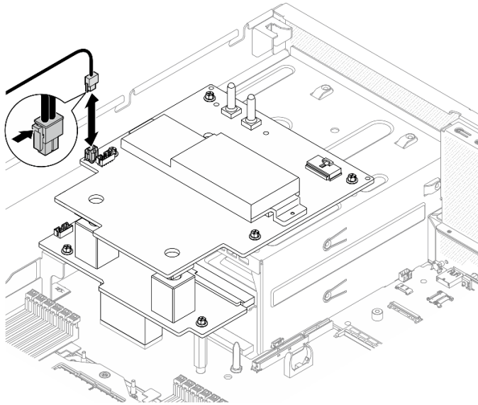
圖例 273. 拔除 CX-7 支架板電源線
