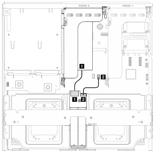
圖例 327. SATA/x4 NVMe M.2 背板纜線佈線 (RAID 配接卡在 PCIe 擴充卡 2 上)
