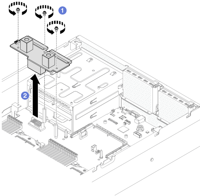
圖例 75. 卸下電源配送板
