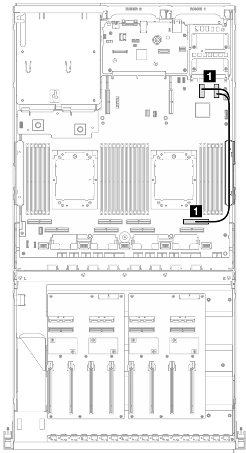
圖例 329. OCP 模組纜線佈線
