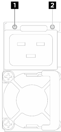
Figura 10. LED de la fuente de alimentación
