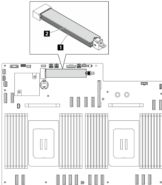
Abbildung 52. M.2-Laufwerksteckplätze
