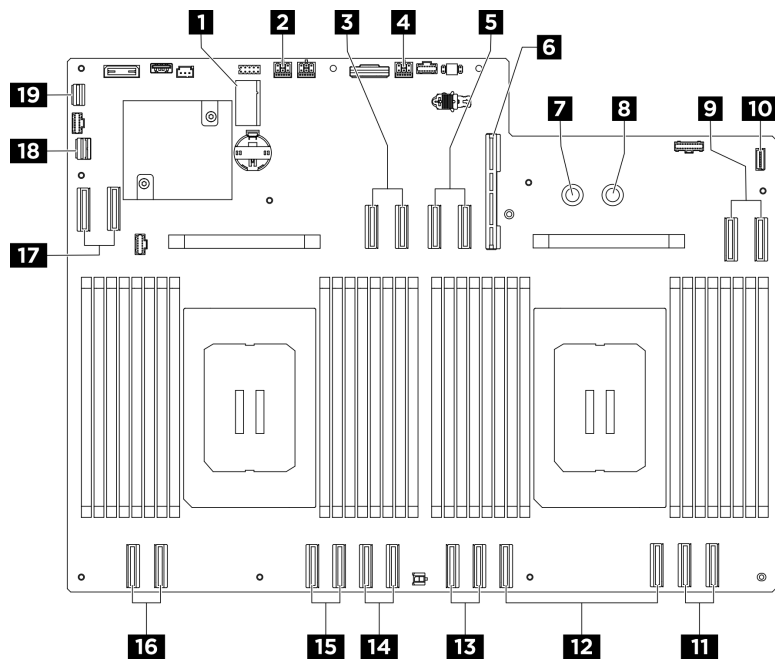
Abbildung 211. Anschlüsse auf der Systemplatine
