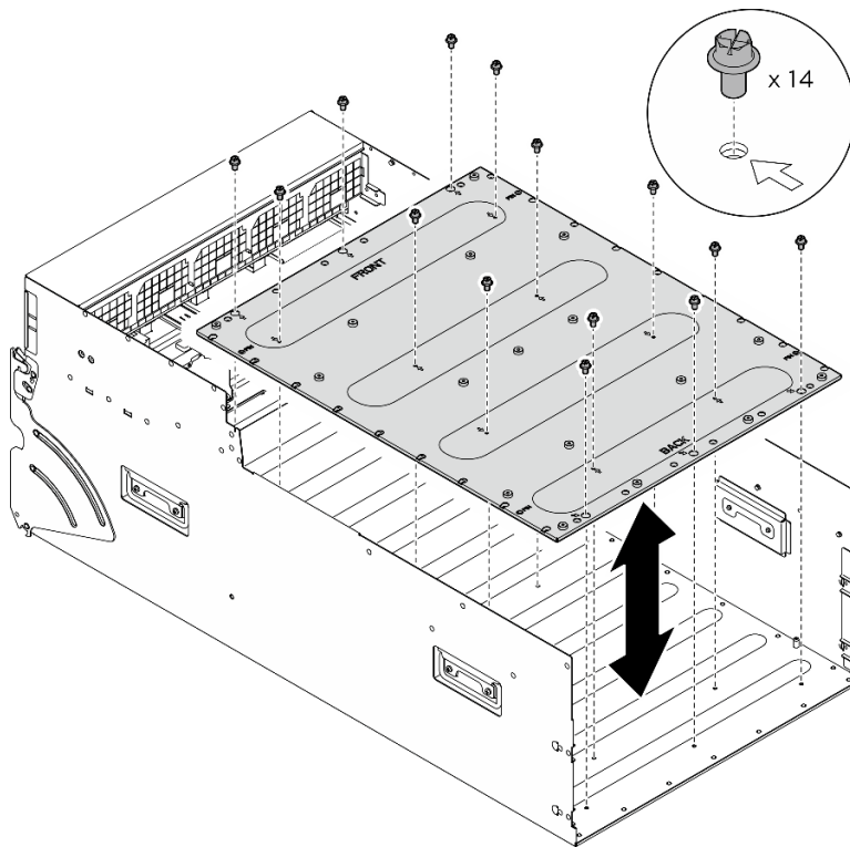
Abbildung 137. Installieren der GPU-Komplex-Adapterplatte
