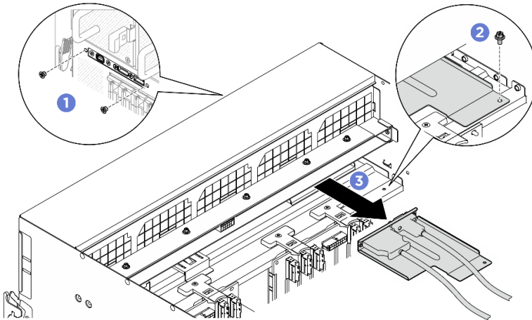
Abbildung 161. Entfernen des E/A-Moduls an der Vorderseite
