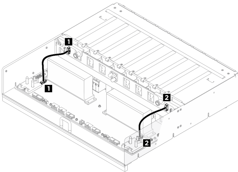
Abbildung 201. Kabelführung für PSU-Interposer
