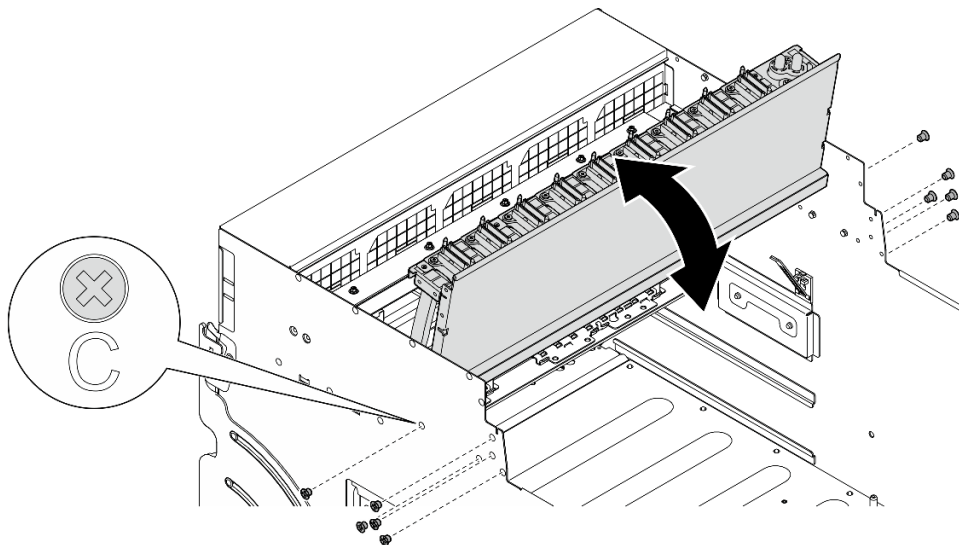
Abbildung 138. Umdrehen des vorderen PCIe-Switch-Kabelbaum
