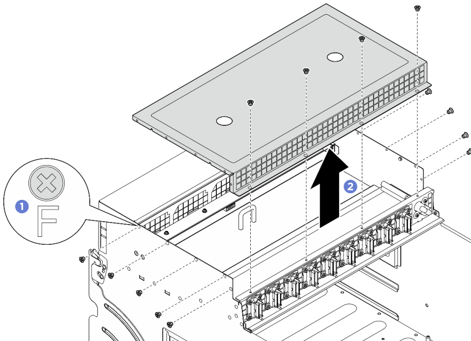
Abbildung 25. Entfernen der Kabelabdeckung
