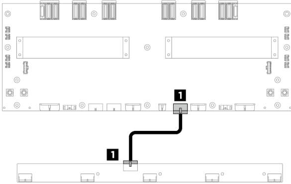
Abbildung 194. Kabelführung für vordere Lüfterplatine
