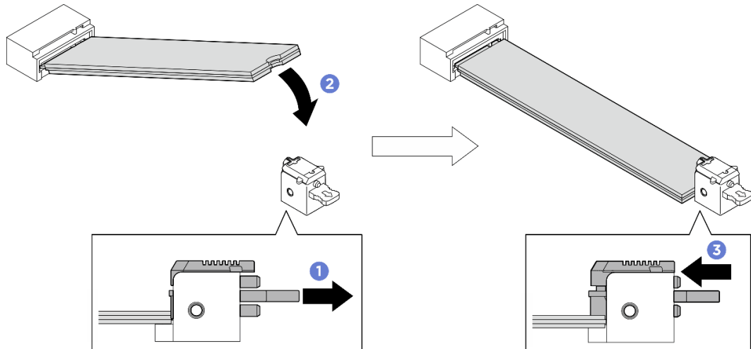
Abbildung 56. Installation des unteren M.2-Laufwerks
