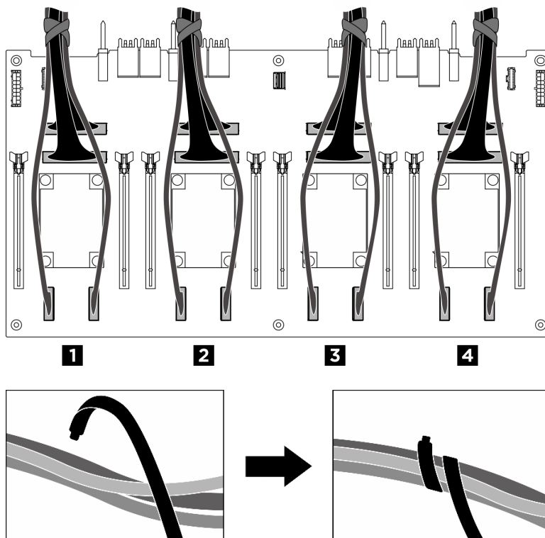
Abbildung 206. Sichern von Kabeln mit Kabelbindern
