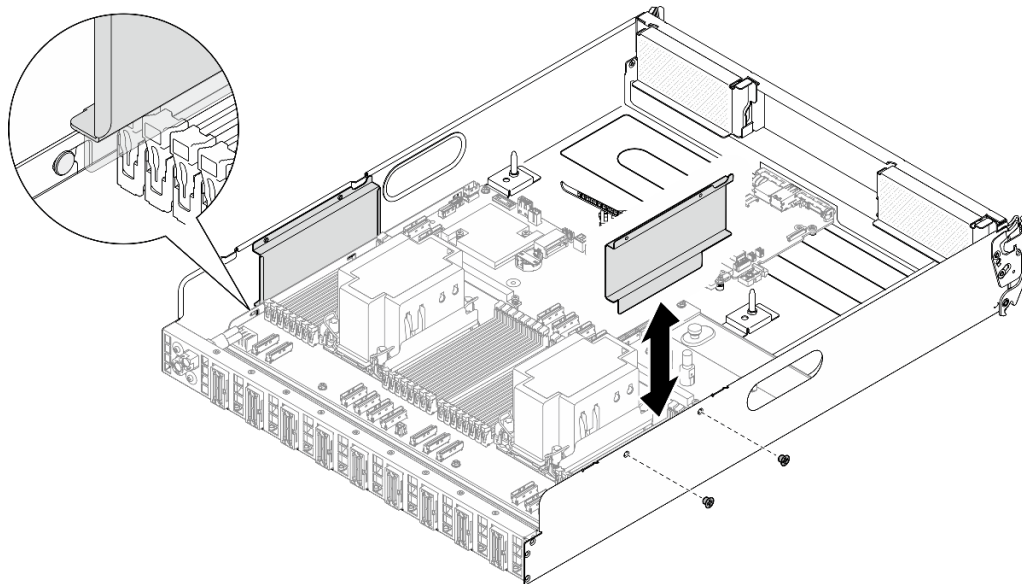
Abbildung 103. Entfernung der Kabelführung
