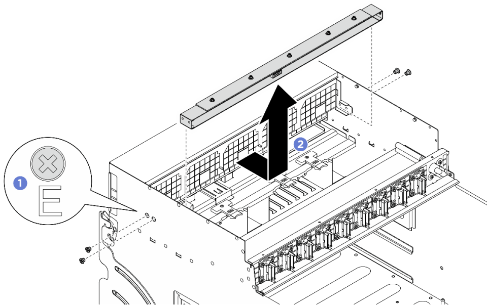
Abbildung 37. Entfernen der vorderen Lüfterplattenbaugruppe
