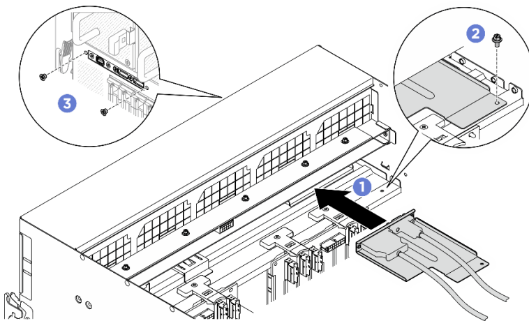
Abbildung 171. Installieren des E/A-Moduls an der Vorderseite
