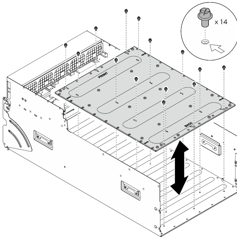
Abbildung 136. Entfernen von GPU-Komplex-Adapterplatte
