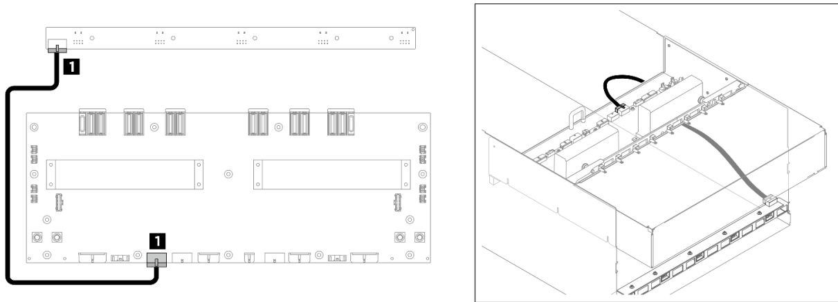
Abbildung 196. Kabelführung für hintere Lüfterplatine (unten)
