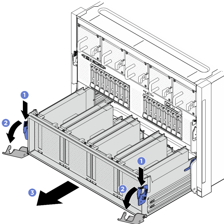
Abbildung 125. Herausziehen des PCIe-Switch-Shuttle bis zum Anschlag
