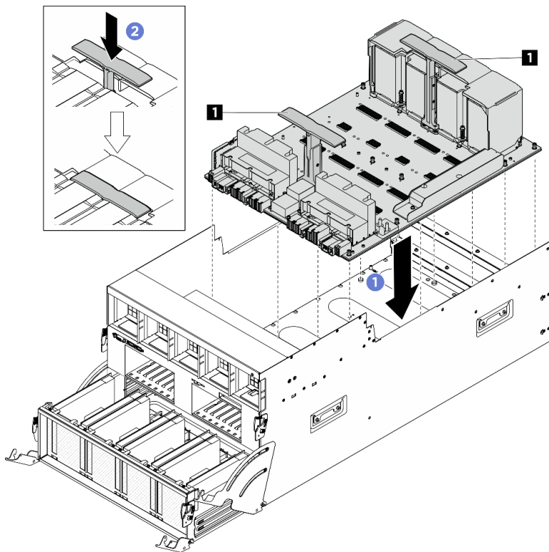
Abbildung 121. Installieren des GPU-Baseboard
