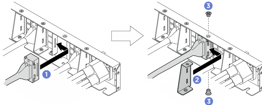
Abbildung 173. Entfernen von Kabel für E/A-Modul an der Vorderseite, integrierte Diagnoseanzeige, GPU-Verwaltung oder Signalkabel
