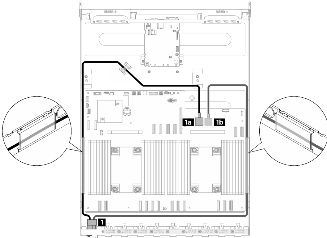
Abbildung 200. Netzkabelführung für Netzkabel
