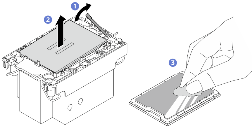
Abbildung 88. Trennen eines Prozessors von Kühlkörper und Träger
