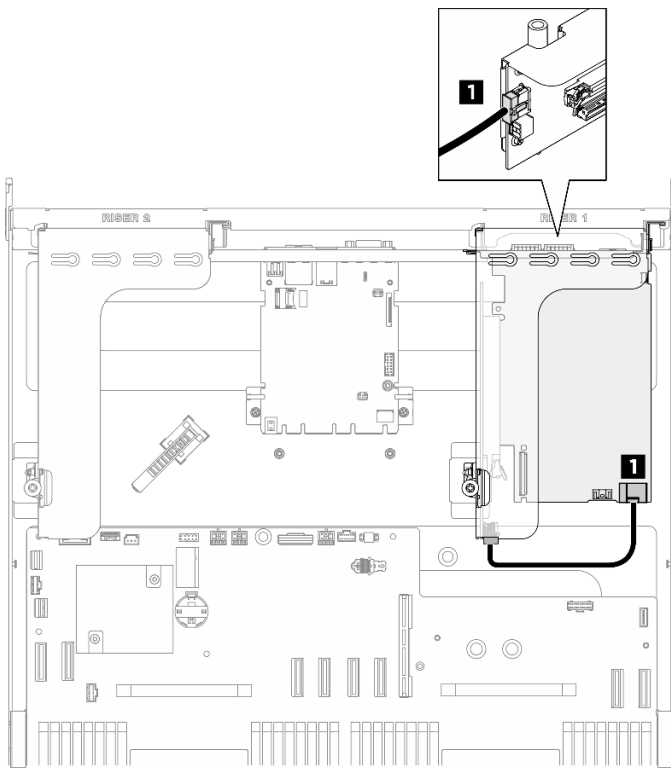
Abbildung 193. DPU-Netzkabelführung
