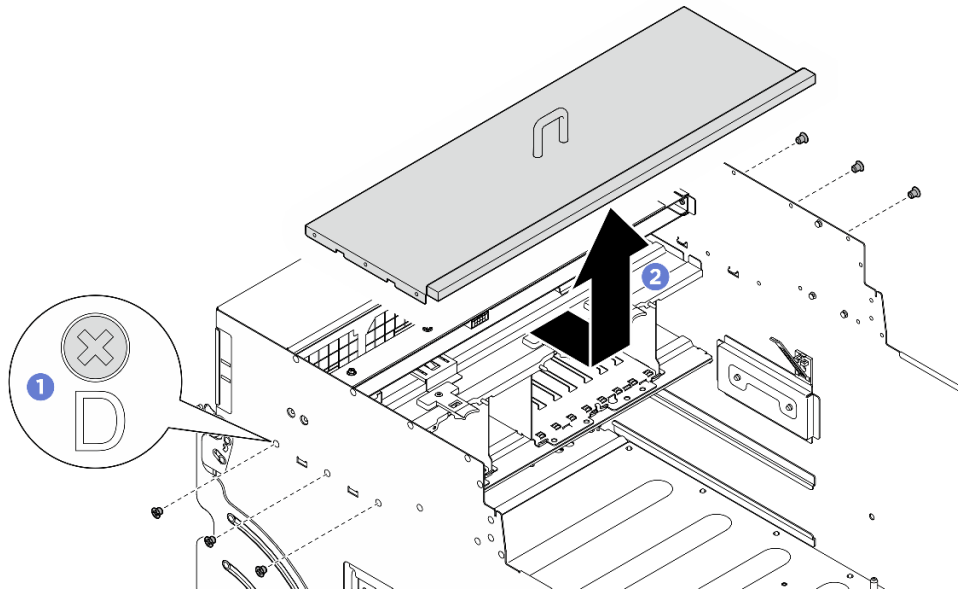
Abbildung 148. Entfernen der E/A-Abdeckung
