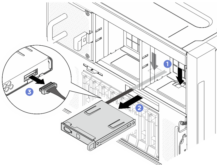
Abbildung 50. Integrierte Diagnoseanzeige entfernen
