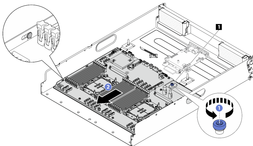
Abbildung 104. Lösen der Systemplatine
