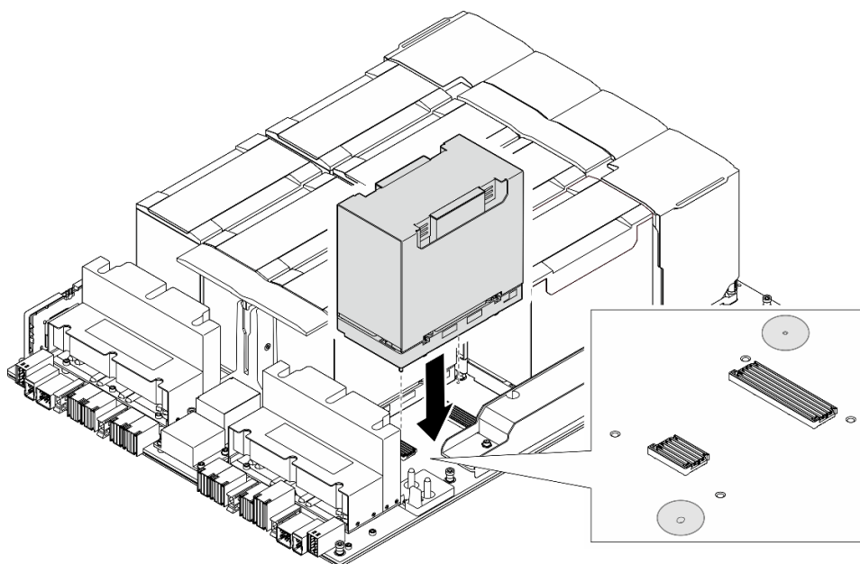
Abbildung 143. Installieren des GPU- und Kühlkörpermodul
