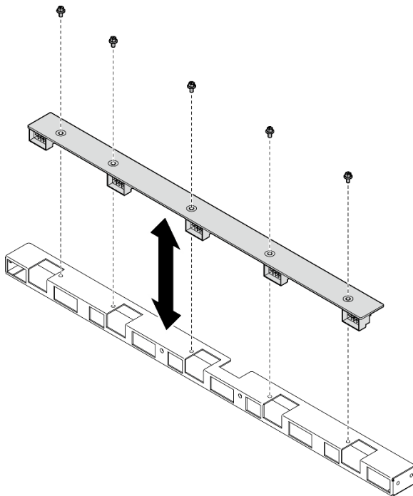
Abbildung 43. Entfernen der hinteren Lüfterplatine
