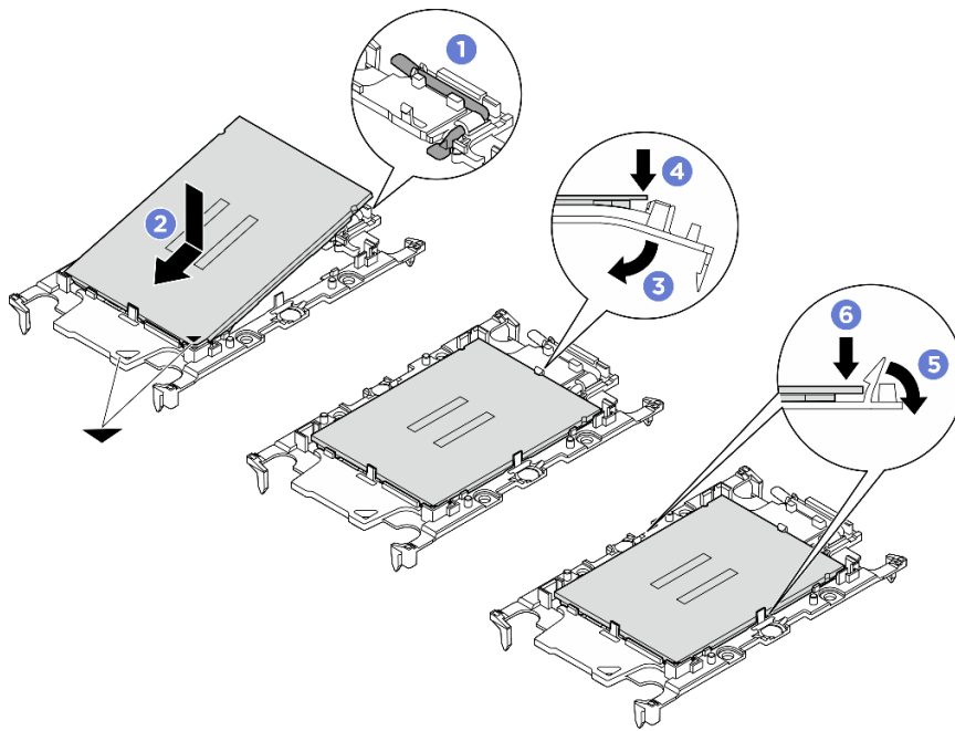
Abbildung 91. Installation des Prozessorträgers
