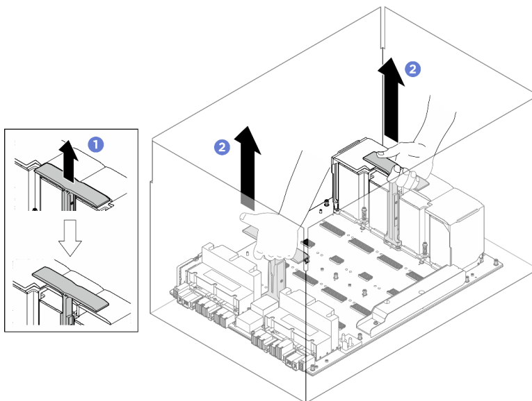
Abbildung 120. Entfernen des GPU-Baseboard aus der Verpackung
