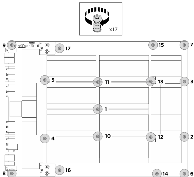
Abbildung 131. Anbringen der Schraube
