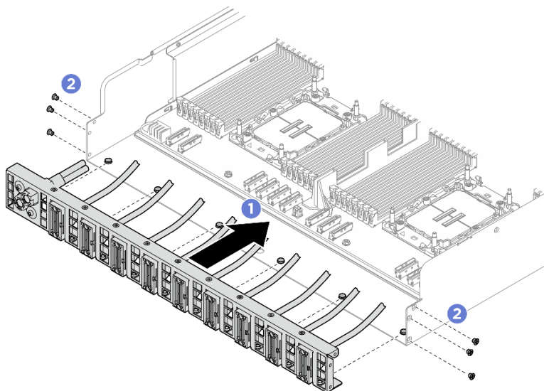
Abbildung 177. Installieren des Hinteren PCIe-Switch-Kabelbaum
