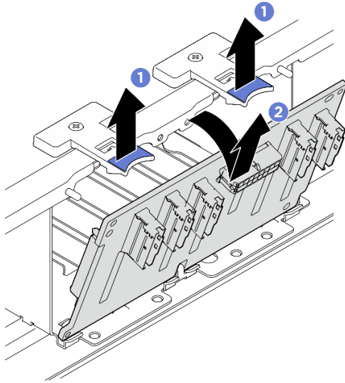
Abbildung 110. Entfernen der Rückwandplatine für 2,5-Zoll-Laufwerke
