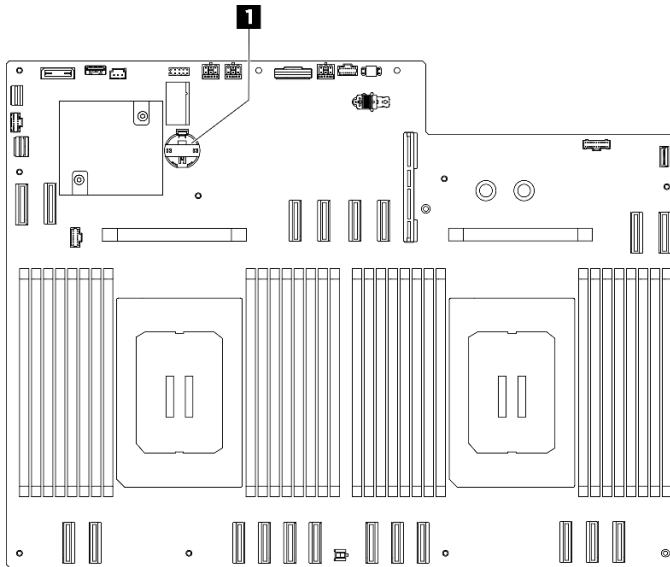
Abbildung 29. Position der CMOS-Batterie
