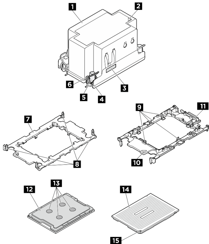
Abbildung 86. PHM-Komponenten
