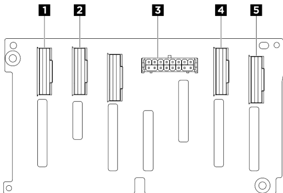
Abbildung 182. Anschlüsse an der 2,5-Zoll-NVMe-Rückwandplatine
