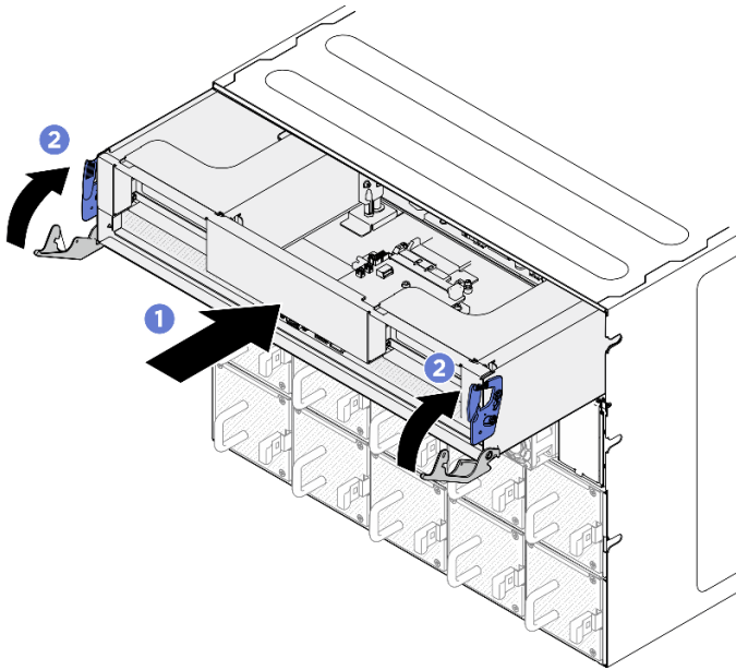
Abbildung 22. Installieren des 2U-Compute-Shuttle
