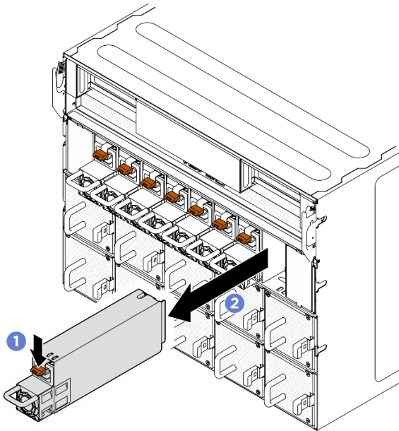
Abbildung 78. Entfernen der Netzteilereinheit
