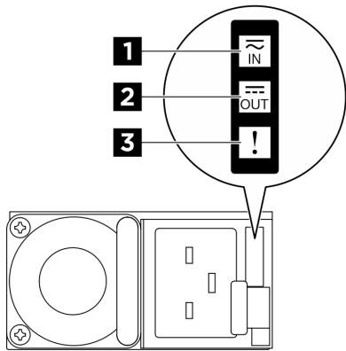
Abbildung 213. CFFv4 Netzteilanzeigen
