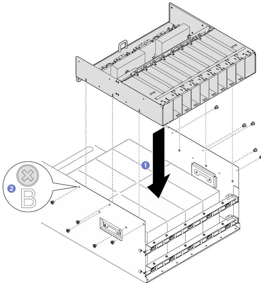
Abbildung 72. Installieren des Stromversorgungskomplex
