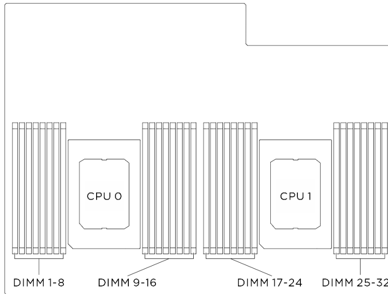
Abbildung 58. Layout für Speichermodule und Prozessoren
