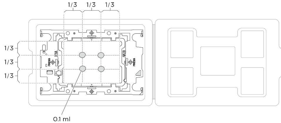
Abbildung 92. Auftragen von Wärmeleitpaste mit Prozessor im Versandeinbaurahmen
