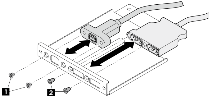
Abbildung 170. Installieren der Kabel des E/A-Moduls an der Vorderseite
