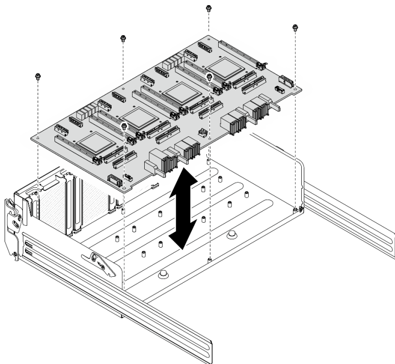
Abbildung 152. Installieren des PCIe-Switch-Platine
