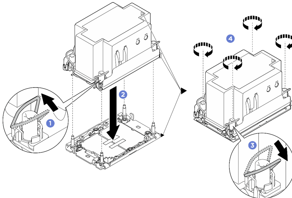
Abbildung 94. Installation des PHM
