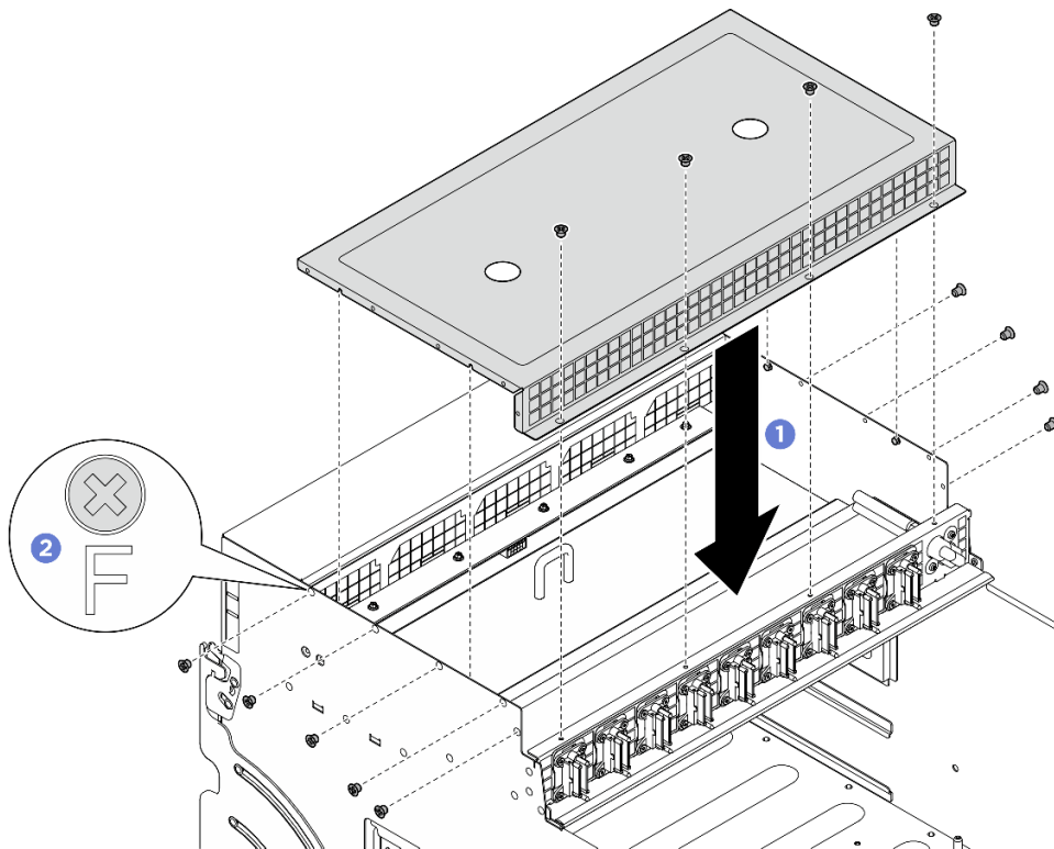
Abbildung 26. Installation der Kabelabdeckung
