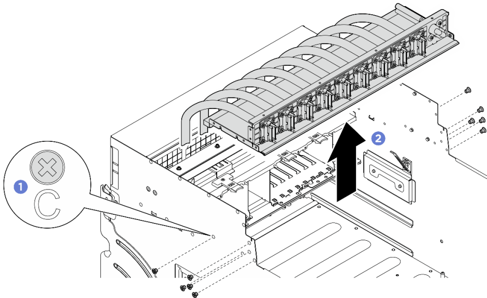
Abbildung 163. Entfernen des Vorderen PCIe-Switch-Kabelbaum
