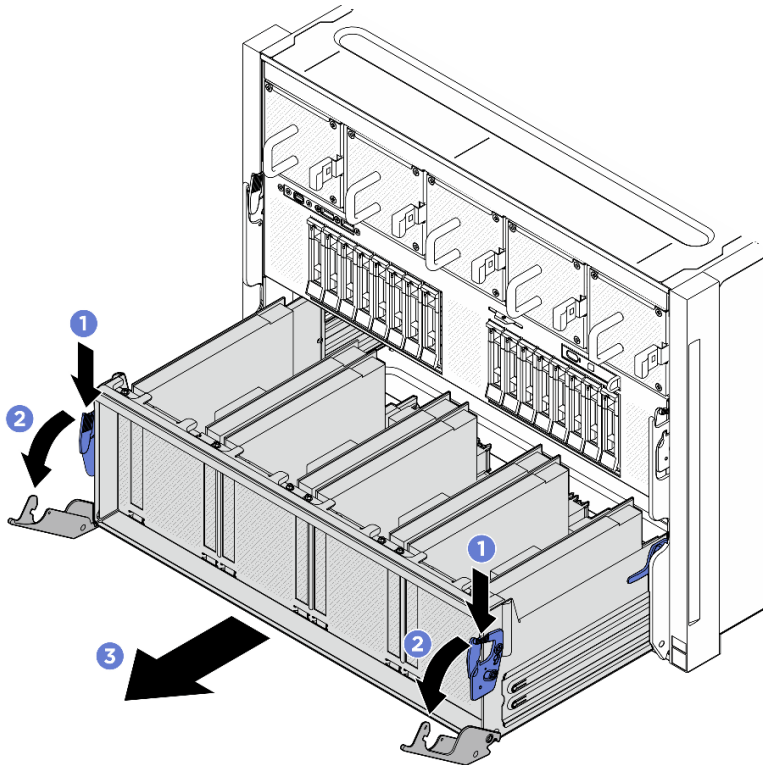
Abbildung 116. Herausziehen des PCIe-Switch-Shuttle bis zum Anschlag
