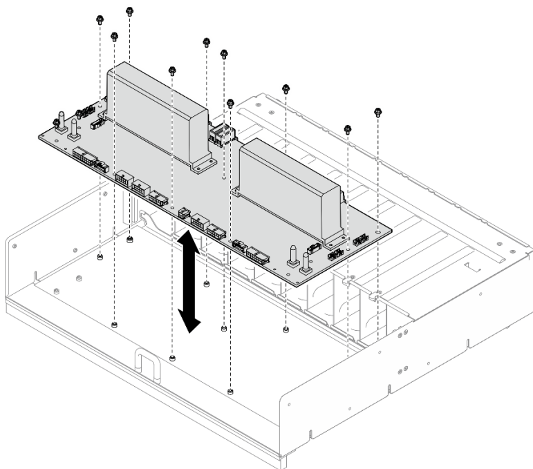
Abbildung 74. Entfernen der Stromversorgungsplatine
