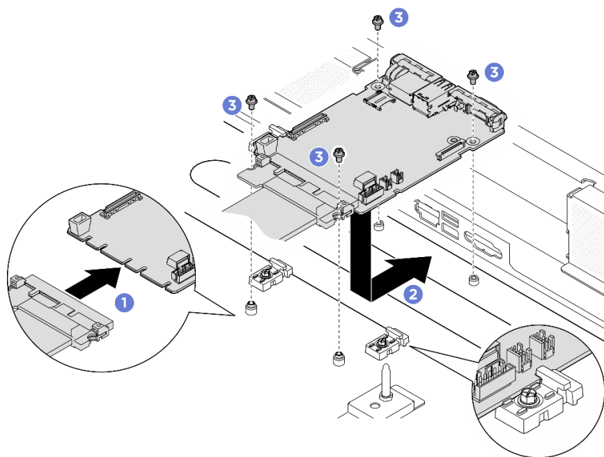
Abbildung 84. Installation der System-E/A-Platine
