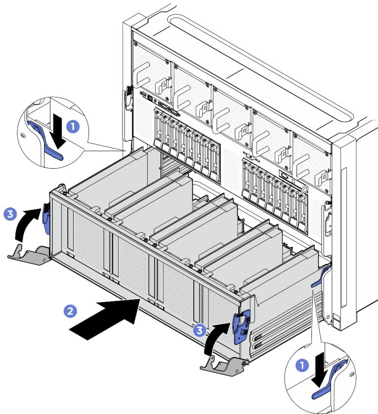
Abbildung 133. Installieren des PCIe-Switch-Shuttle im 8U-GPU-Shuttle
