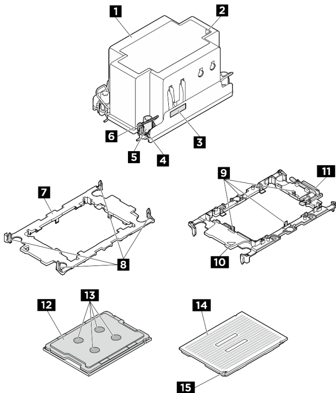
Abbildung 85. PHM-Komponenten
