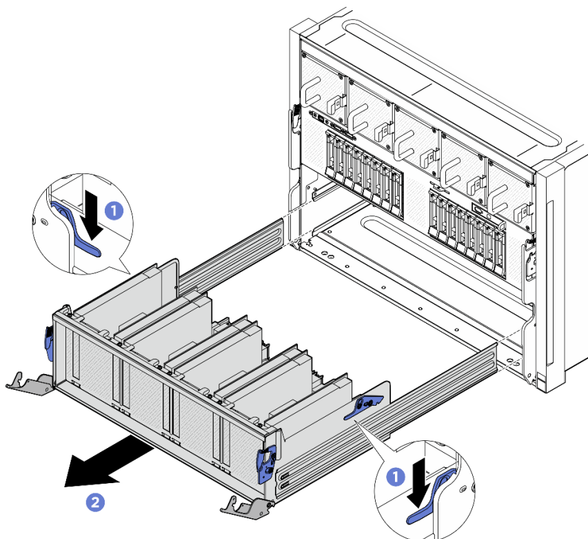
Abbildung 179. Entfernen des PCIe-Switch-Shuttle aus dem 8U-GPU-Shuttle
