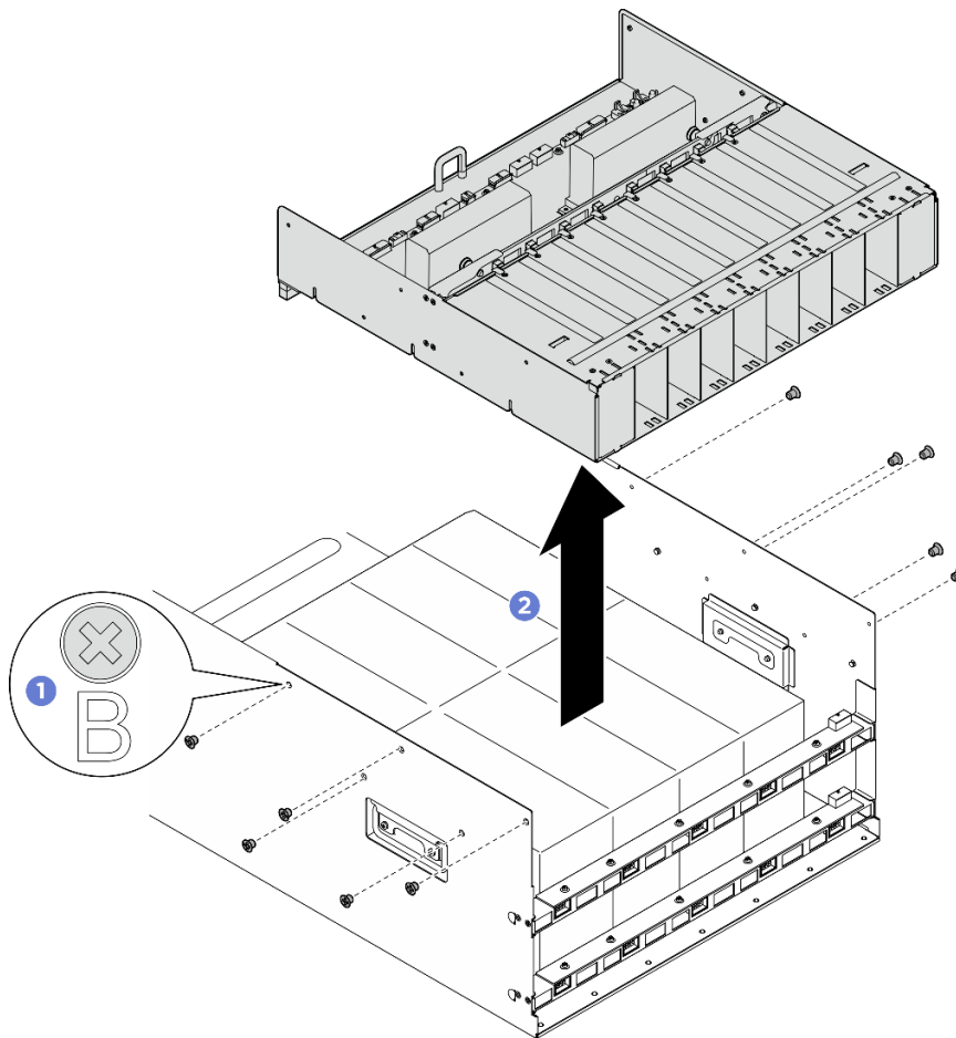
Abbildung 71. Entfernen des Stromversorgungskomplex
