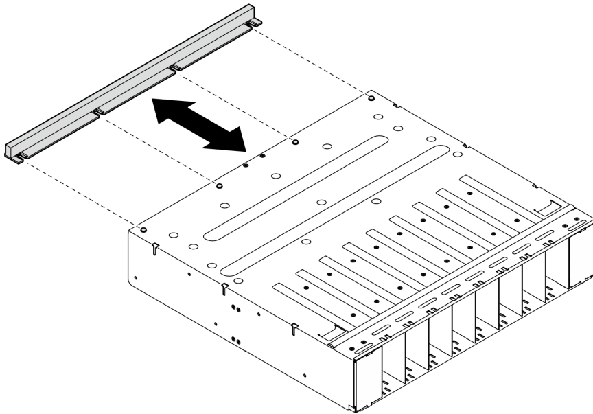
Abbildung 49. Installation der GPU-Luftführung
