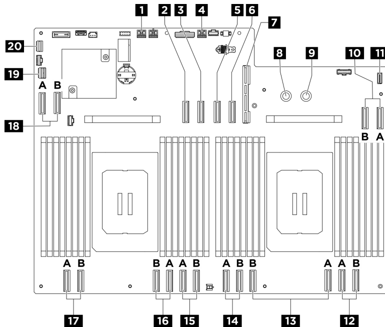
Abbildung 191. Anschlüsse auf der Systemplatine für die Kabelführung
