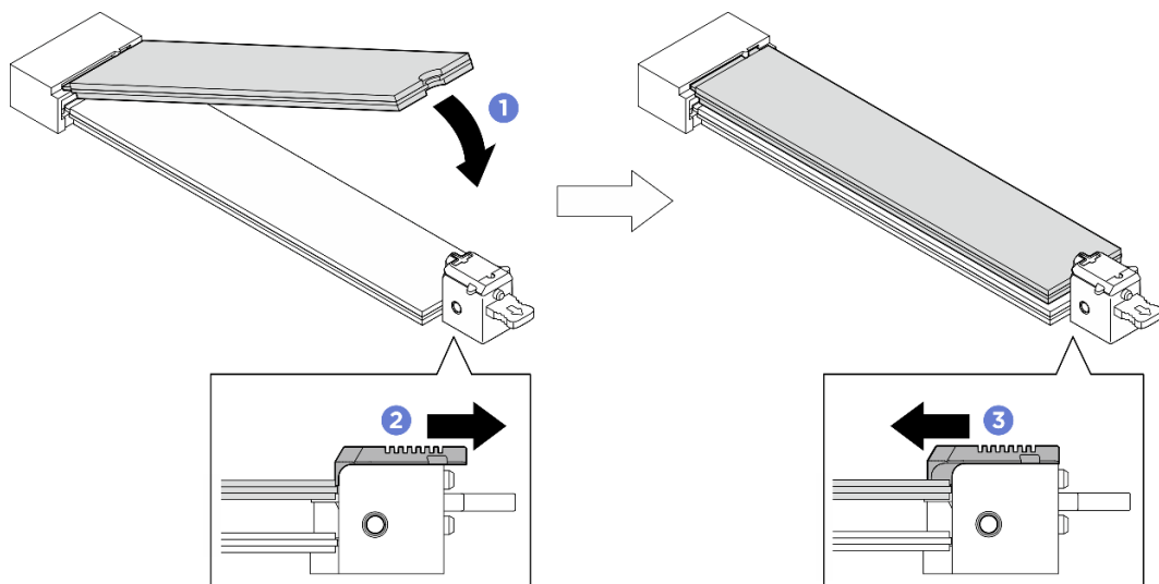
Abbildung 57. Installation des oberen M.2-Laufwerks
