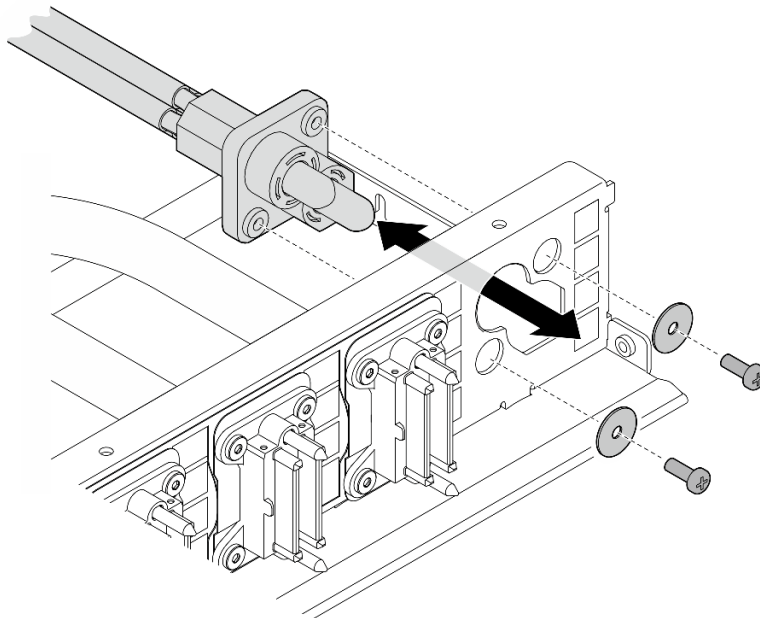
Abbildung 165. Entfernen des Netzkabels
