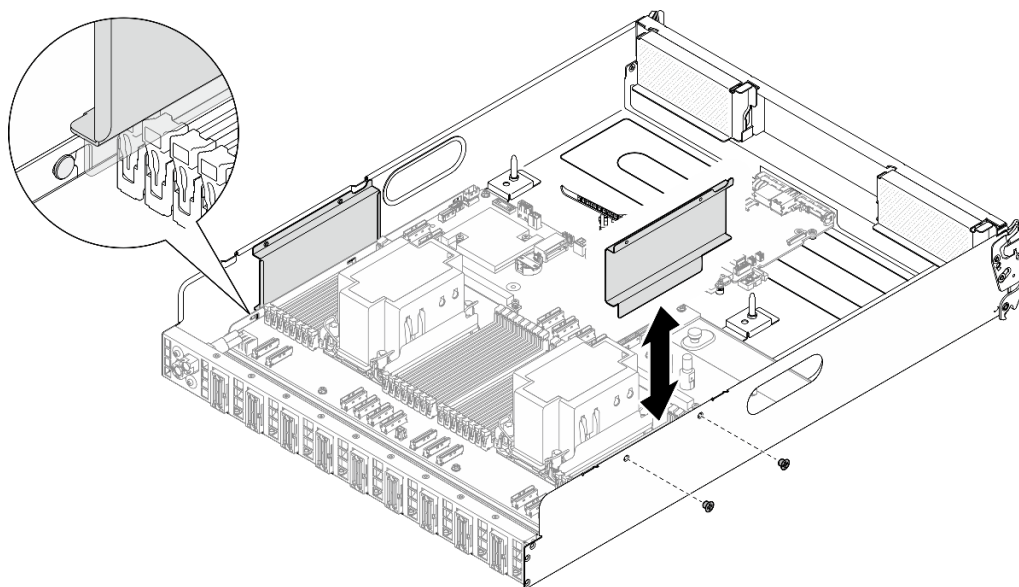
Abbildung 108. Installation der Kabelführung
