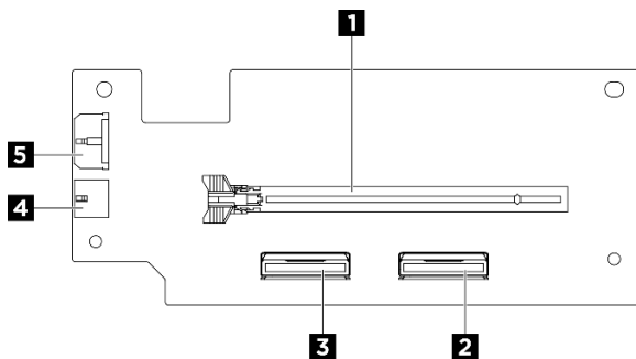
Abbildung 185. Anschlüsse an der PCIe-Adapterkarte
