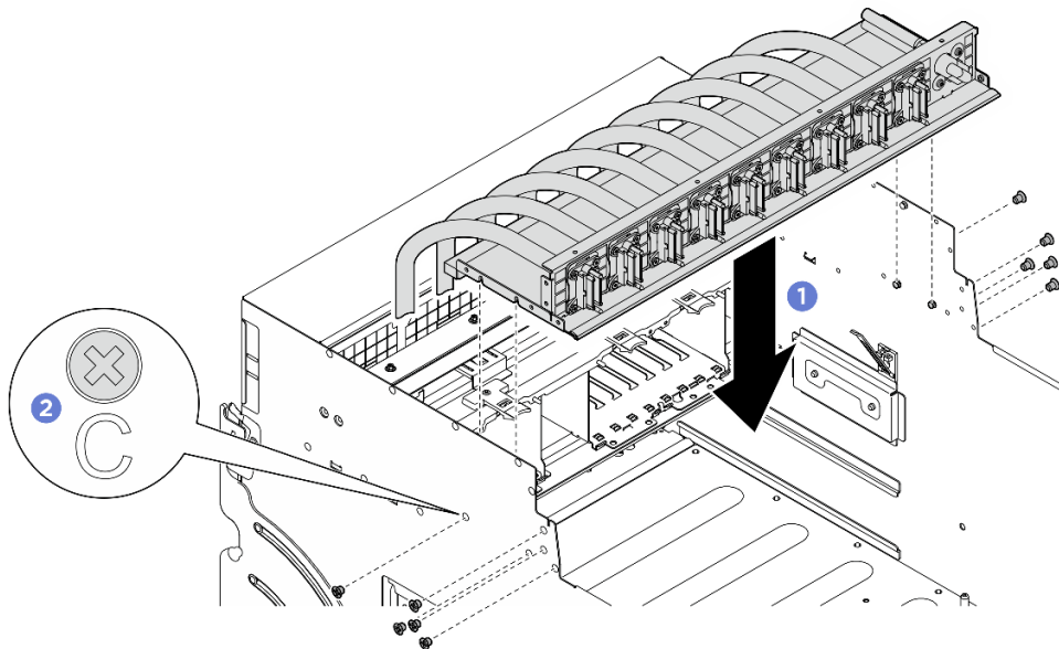
Abbildung 169. Installieren des Vorderen PCIe-Switch-Kabelbaum
