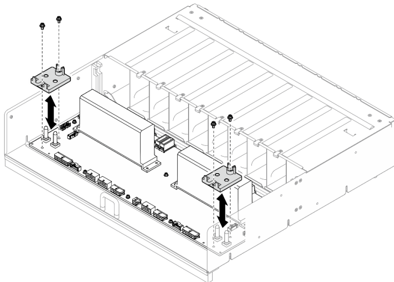
Abbildung 73. Kabelhalterklammer entfernen
