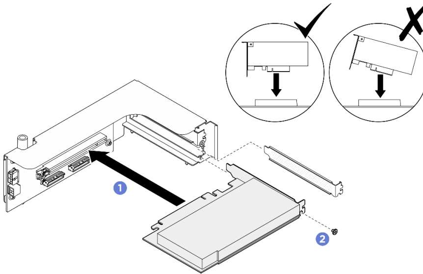
Abbildung 160. Installation des hinteren PCIe-Adapters
