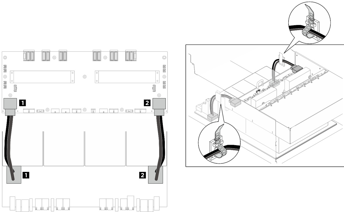
Abbildung 205. Kabelführung für GPU-Baseboard
