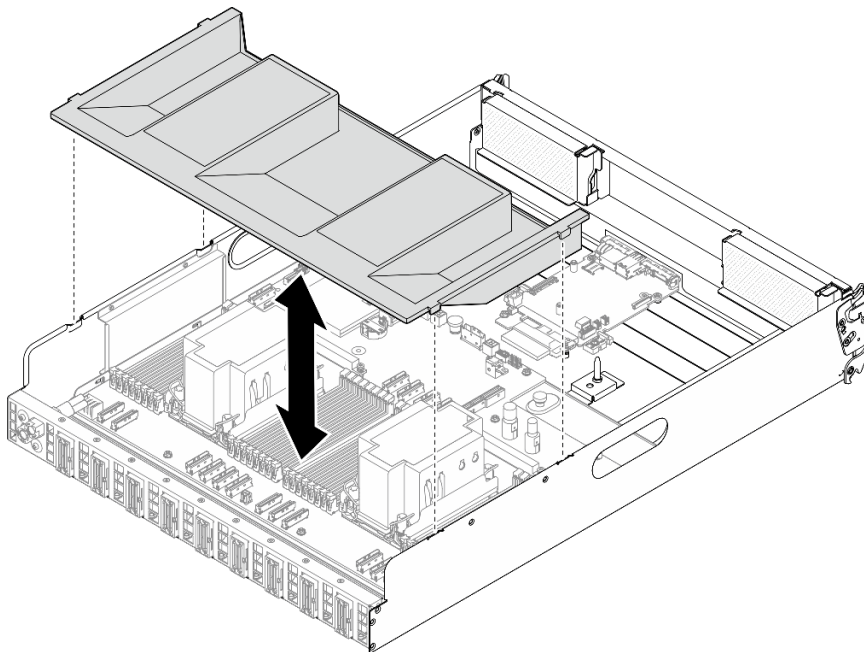
Abbildung 82. Installation der Prozessorluftführung
