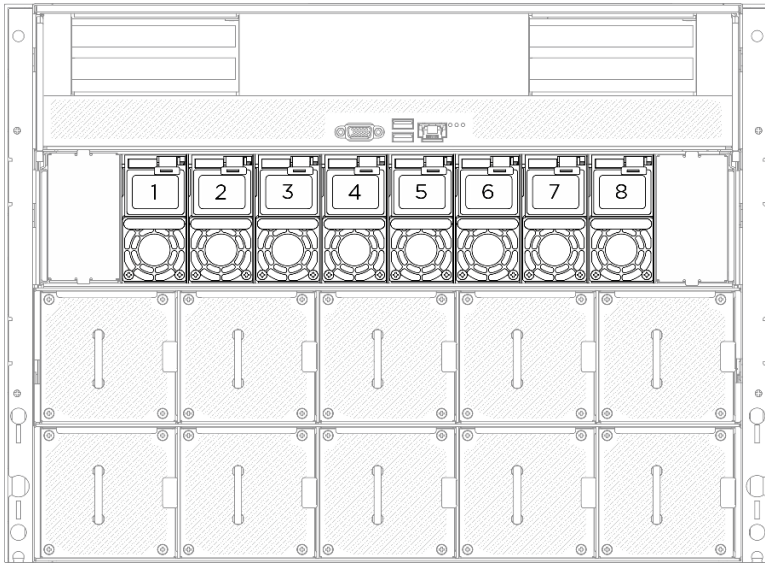
Abbildung 77. Nummerierung der Netzteilpositionen
