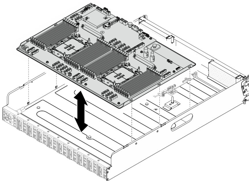
Abbildung 105. Entfernen der Systemplatine
