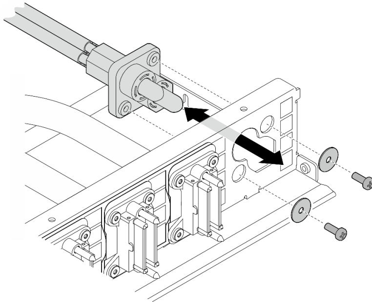
Abbildung 168. Installieren des Netzkabels
