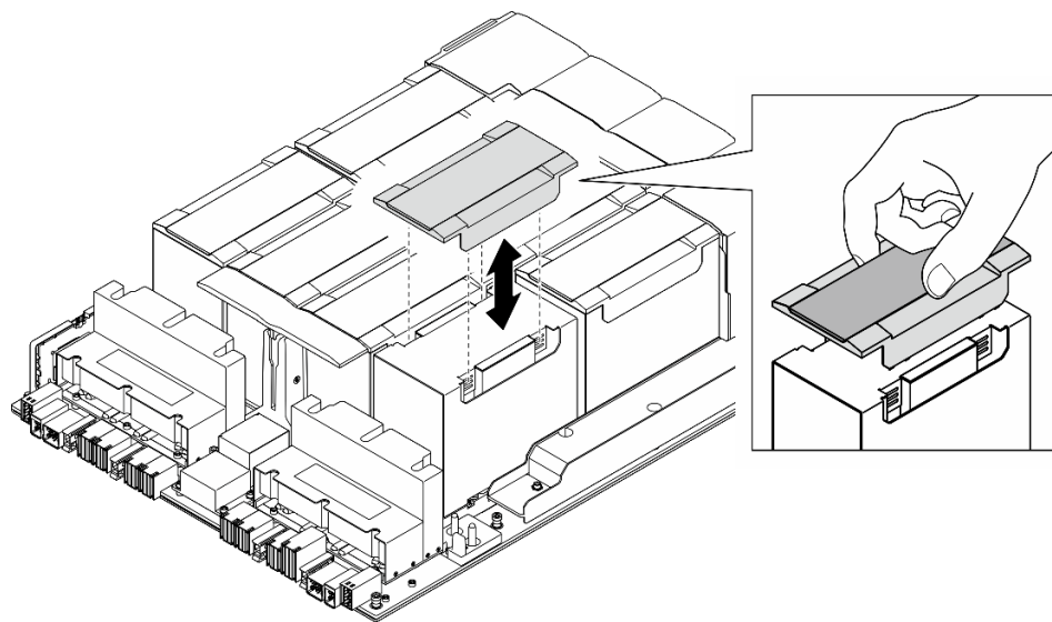
Abbildung 142. Entfernen der Kunststoffabdeckung
