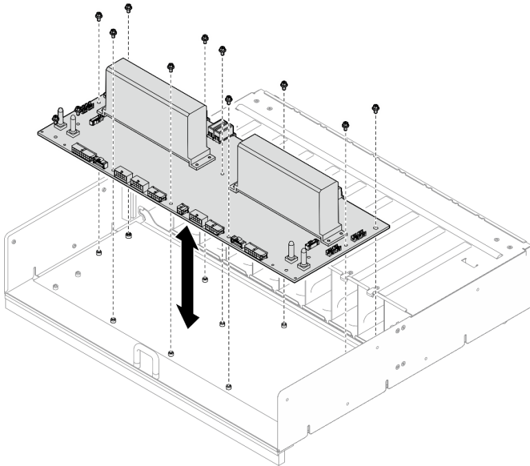
Abbildung 75. Installation der Stromversorgungsplatine
