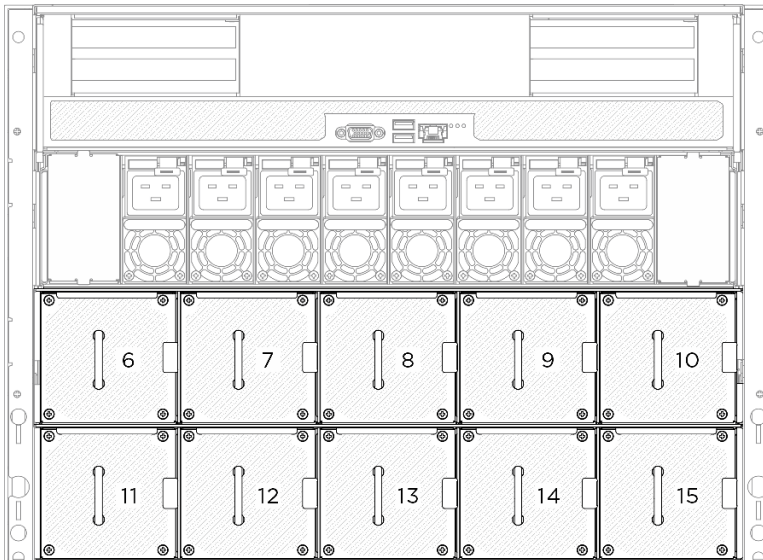
Abbildung 32. Nummerierung der hinteren Lüfter
