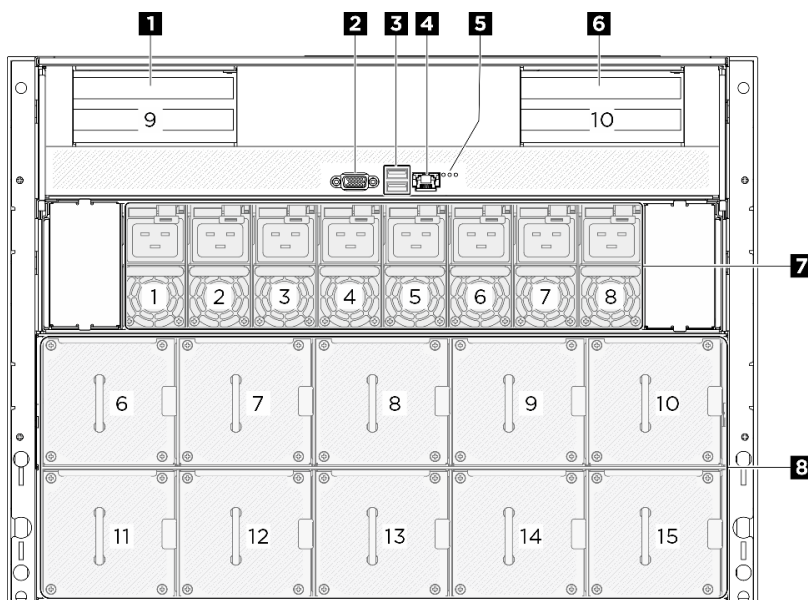
Abbildung 4. Rückansicht
