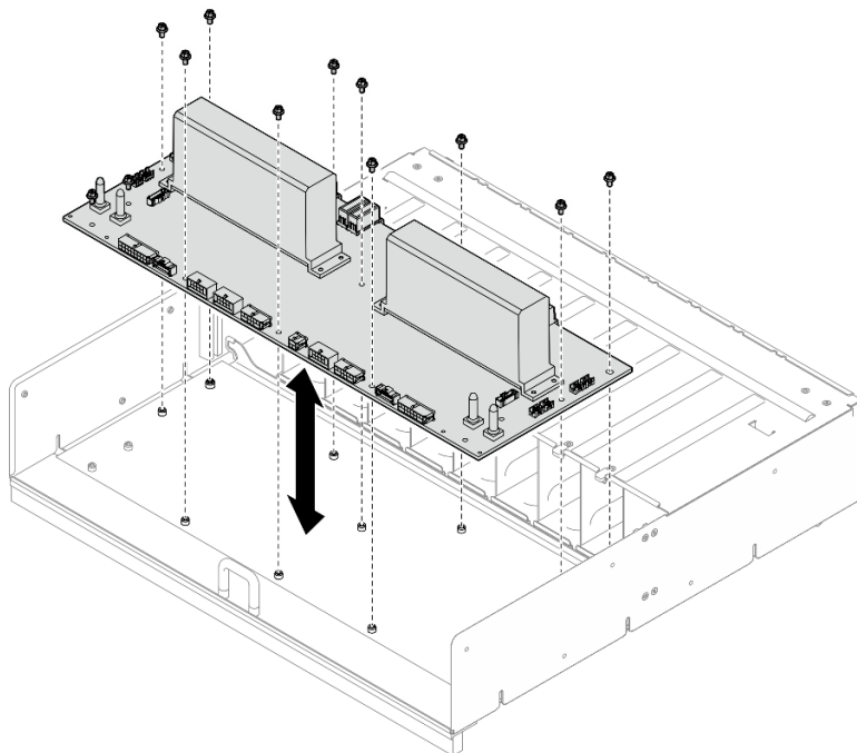
Figura 98. Installazione della scheda di distribuzione dell'alimentazione
