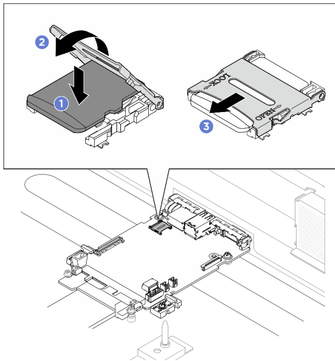
Figura 63. Installazione della scheda MicroSD
