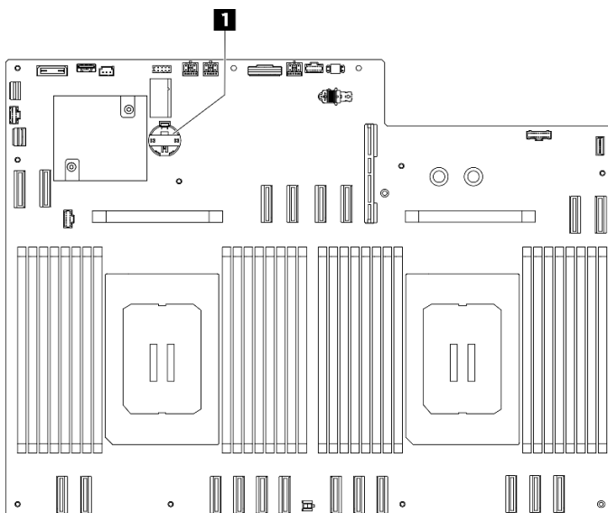
Figura 29. Posizione della batteria CMOS
