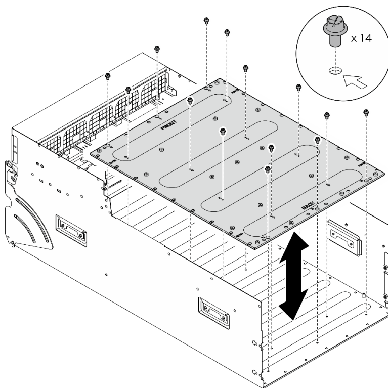
Figura 136. Rimozione della Piastra adattatore del complesso GPU
