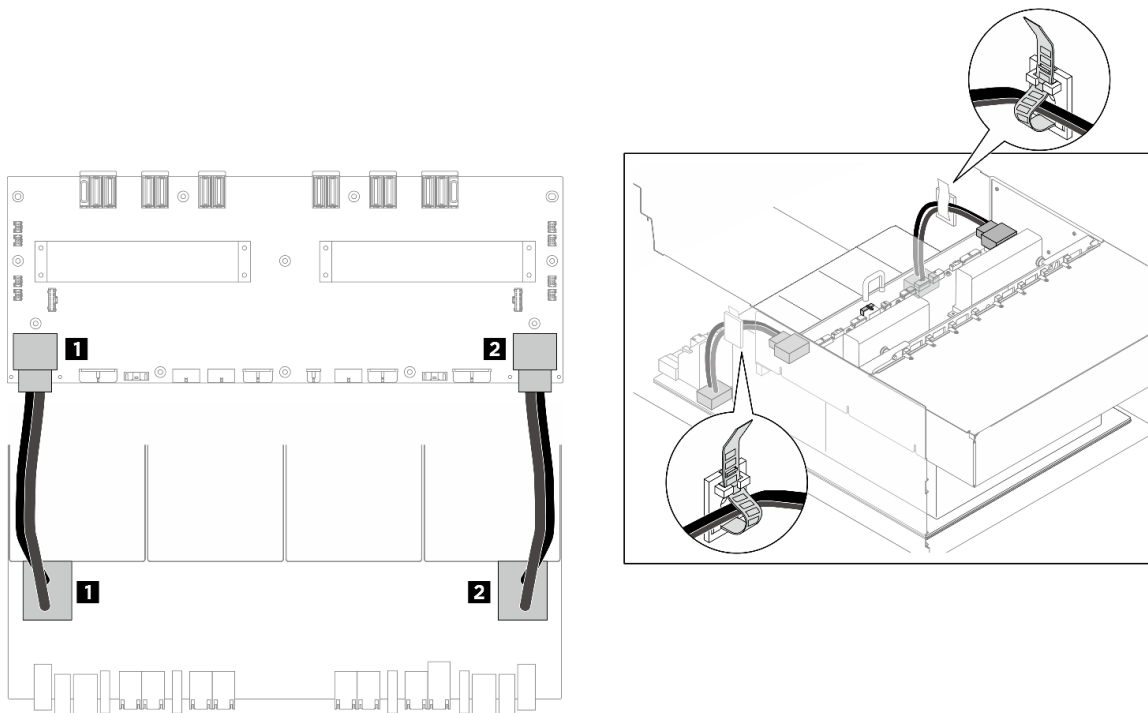
Figura 205. Instradamento dei cavi per la Scheda di base GPU
