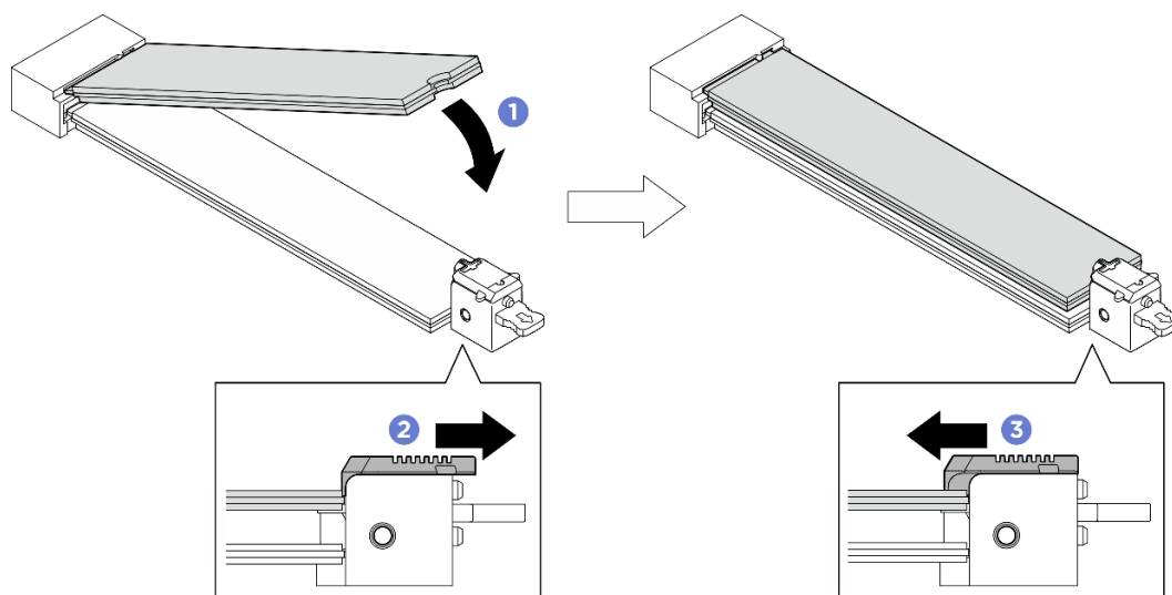
Figura 57. Installazione dell'unità M.2 superiore
