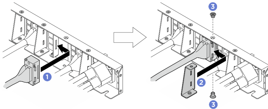
Figura 173. Rimozione del cavo per modulo I/O anteriore, pannello di diagnostica integrato, gestione GPU o segnale
