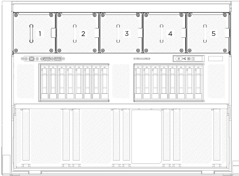
Figura 34. Numerazione delle ventole anteriori
