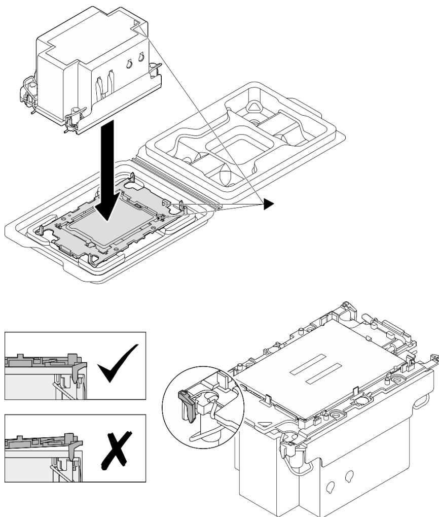
Figura 93. Assemblaggio del PHM con il processore nella confezione di spedizione
