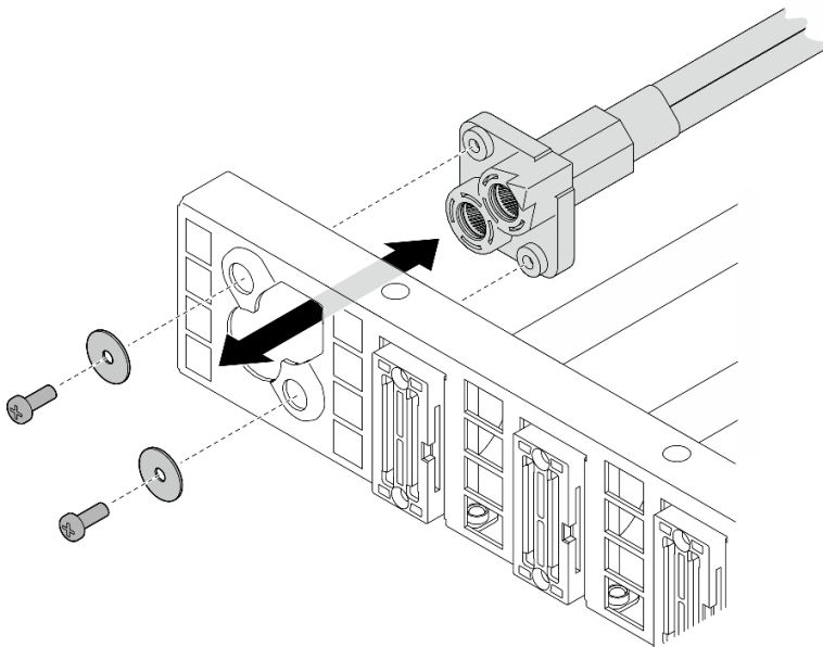
Figura 174. Rimozione del cavo di alimentazione
