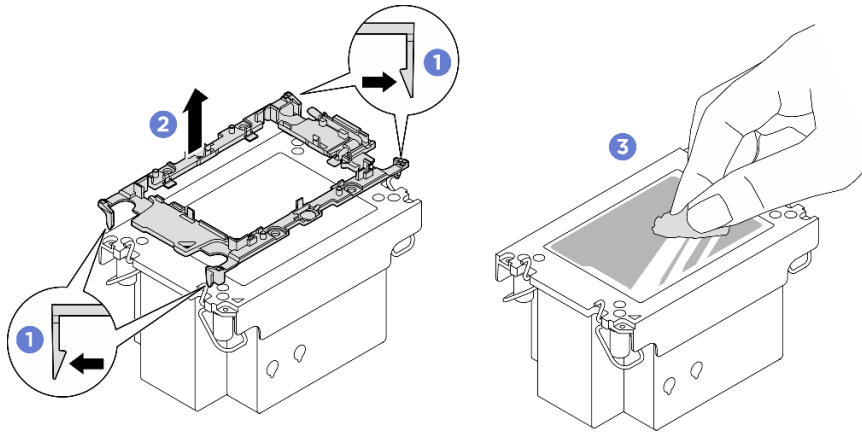
Figura 89. Separazione di una piastra del processore dal dissipatore di calore
