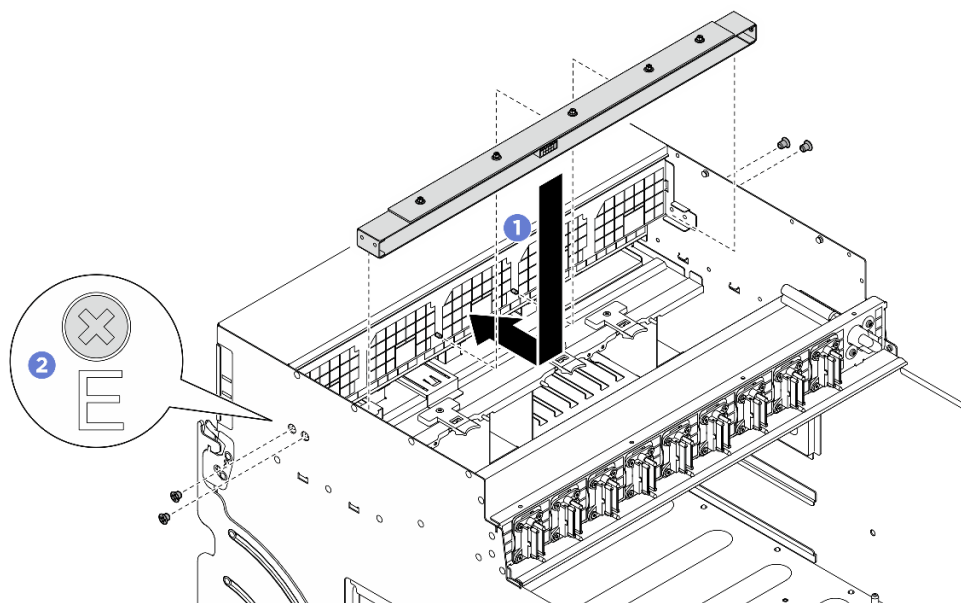
Figura 40. Installazione dell'assieme della scheda di controllo della ventola anteriore
