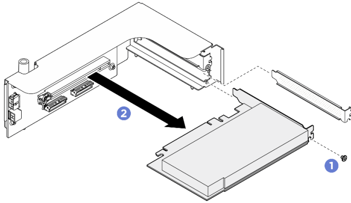
Figura 159. Rimozione dell'adattatore PCIe posteriore
