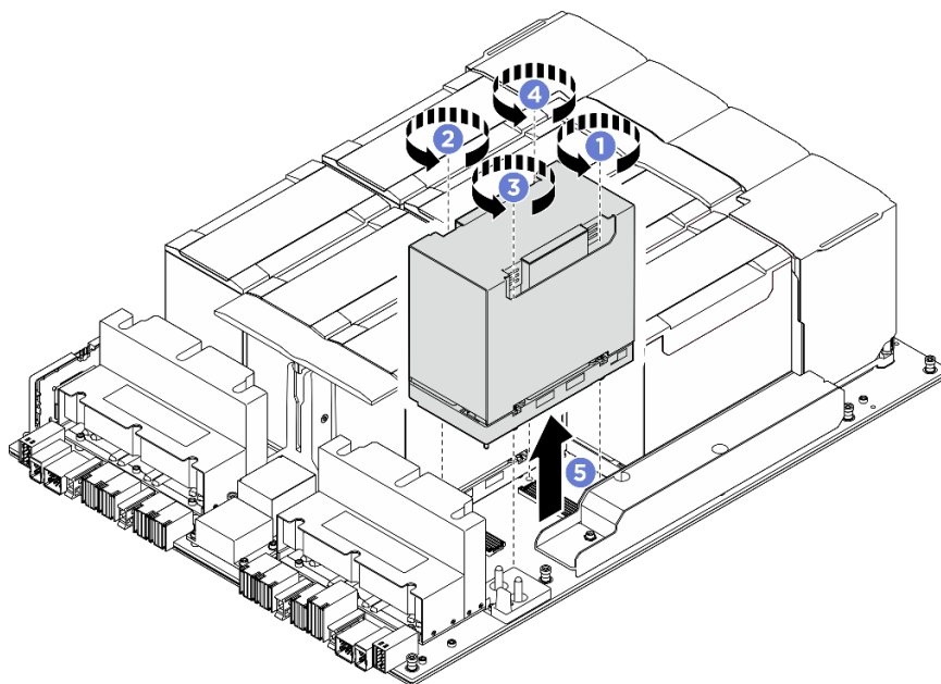
Figura 141. Rimozione del Modulo del dissipatore di calore e GPU
