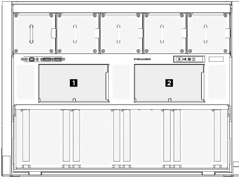
Figura 111. Numerazione dei backplane dell'unità da 2,5"
