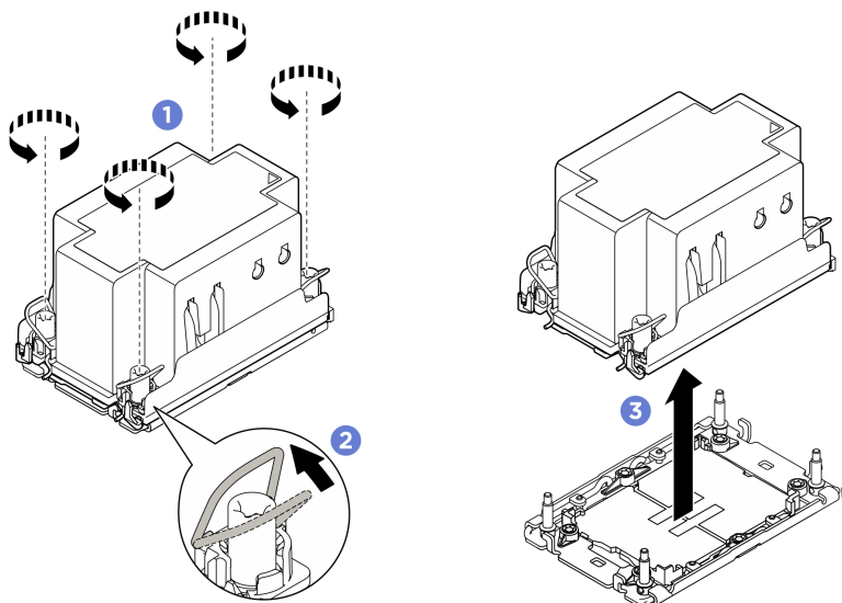
Figura 87. Rimozione del PHM
