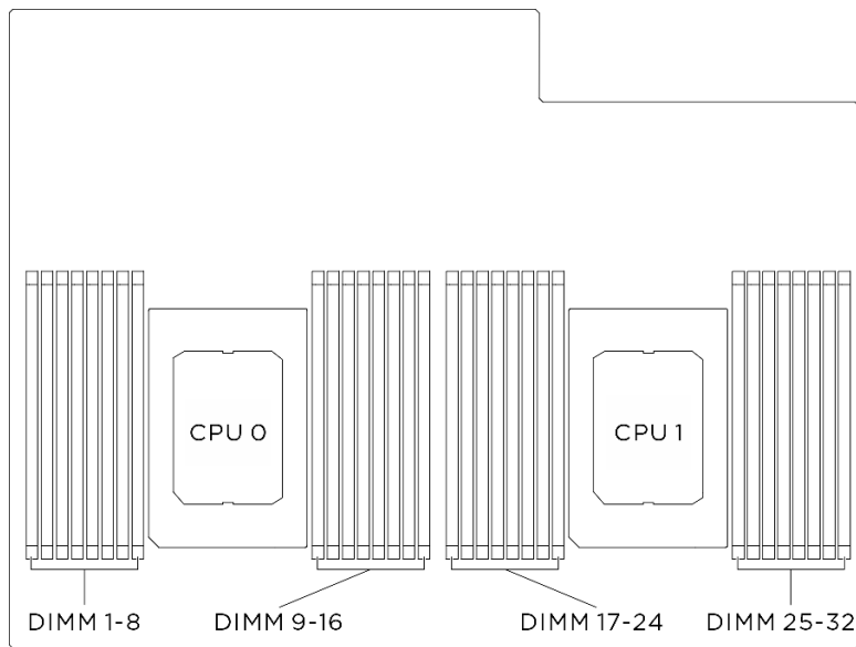
Figura 58. Layout dei moduli di memoria e dei processori
