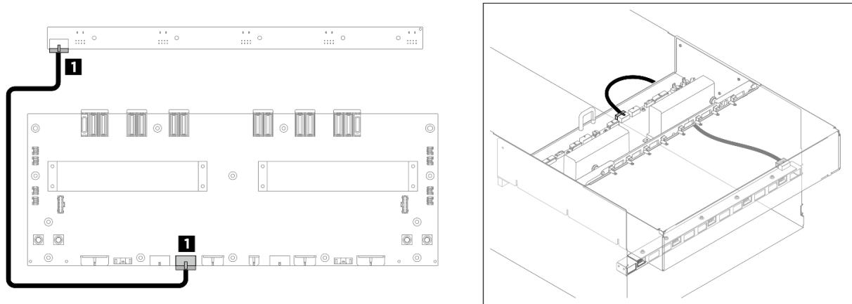
Figura 195. Instradamento dei cavi della scheda di controllo della ventola posteriore (superiore)
