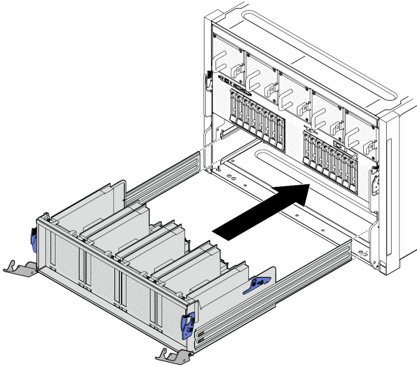
Figura 180. Installazione dello Shuttle dello switch PCIe in posizione di blocco
