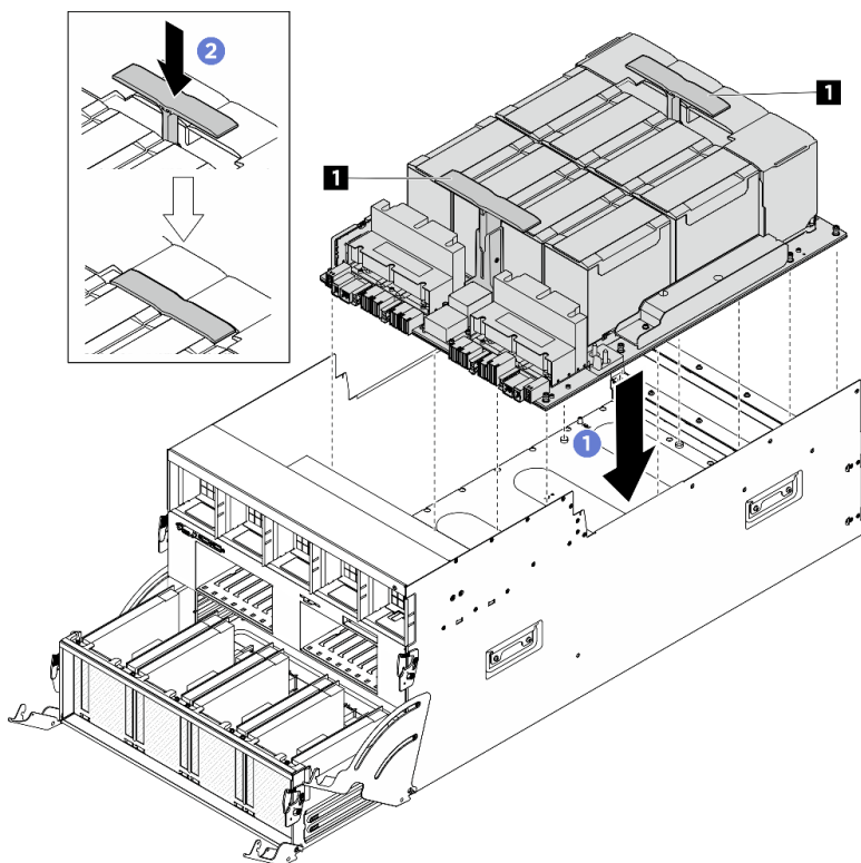
Figura 130. Installazione del Complesso GPU
