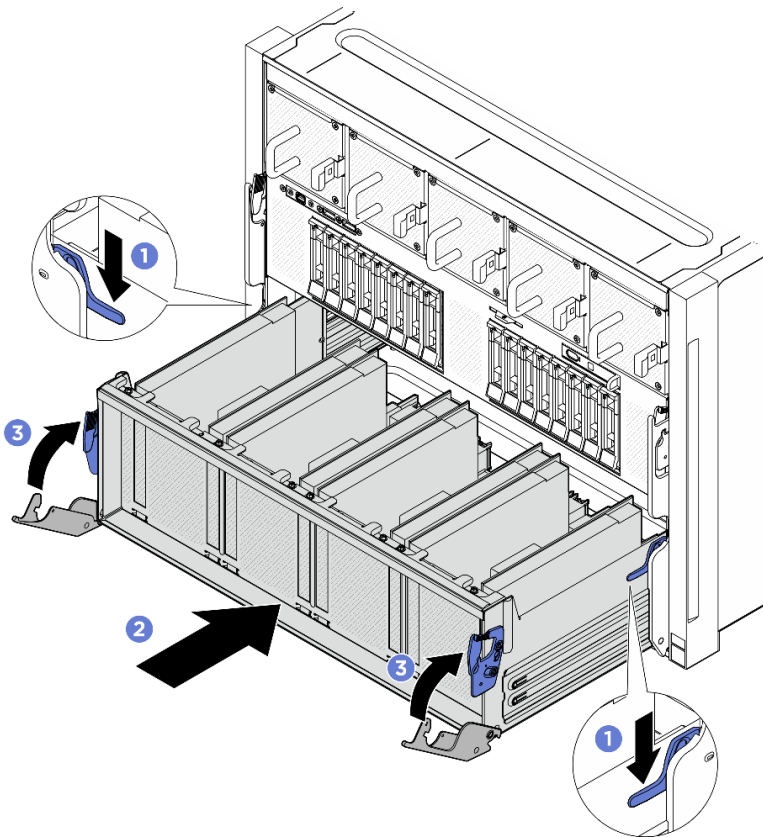
Figura 133. Installazione dello Shuttle dello switch PCIe nello shuttle GPU 8U
