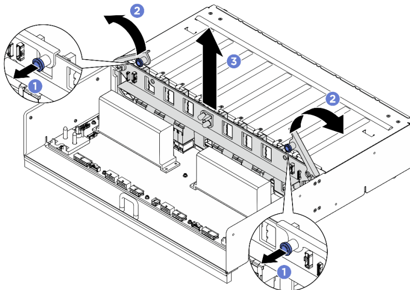
Figura 95. Rimozione del Interposer PSU
