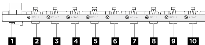
Figura 188. Cavi del cablaggio dello switch PCIe posteriore
