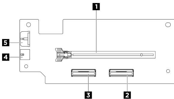
Figura 185. Connettori sulla scheda verticale PCIe
