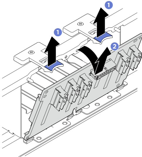
Figura 110. Rimozione del backplane dell'unità da 2,5"
