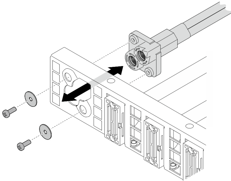
Figura 176. Installazione del cavo di alimentazione
