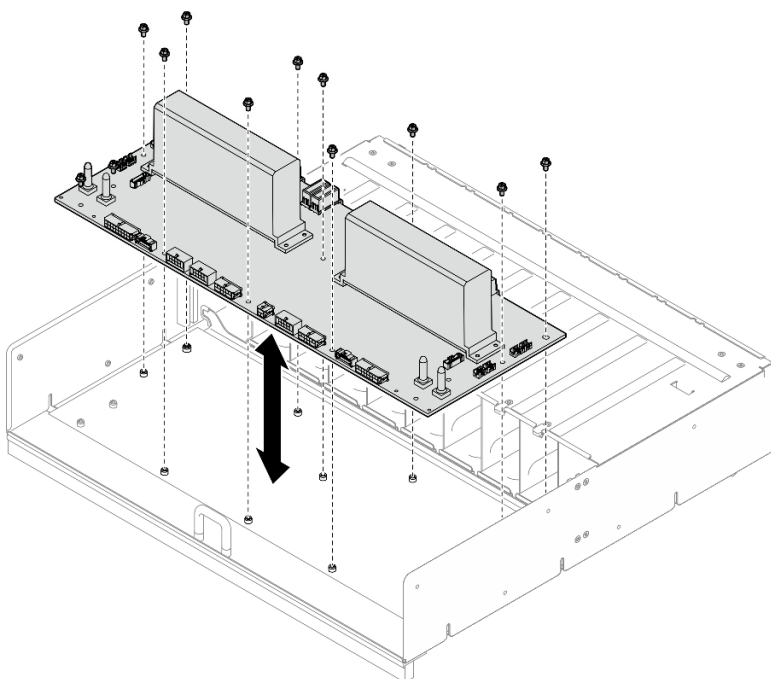
Figura 74. Rimozione della scheda di distribuzione dell'alimentazione
