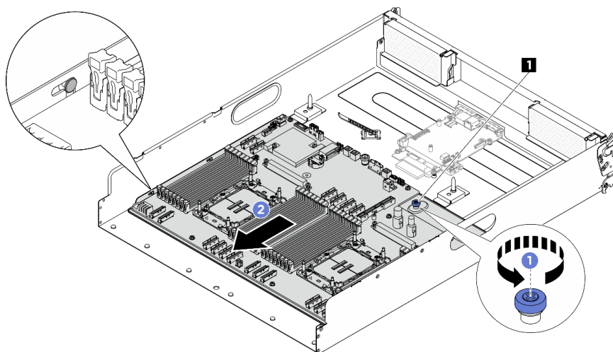
Figura 104. Sganciamento della scheda di sistema
