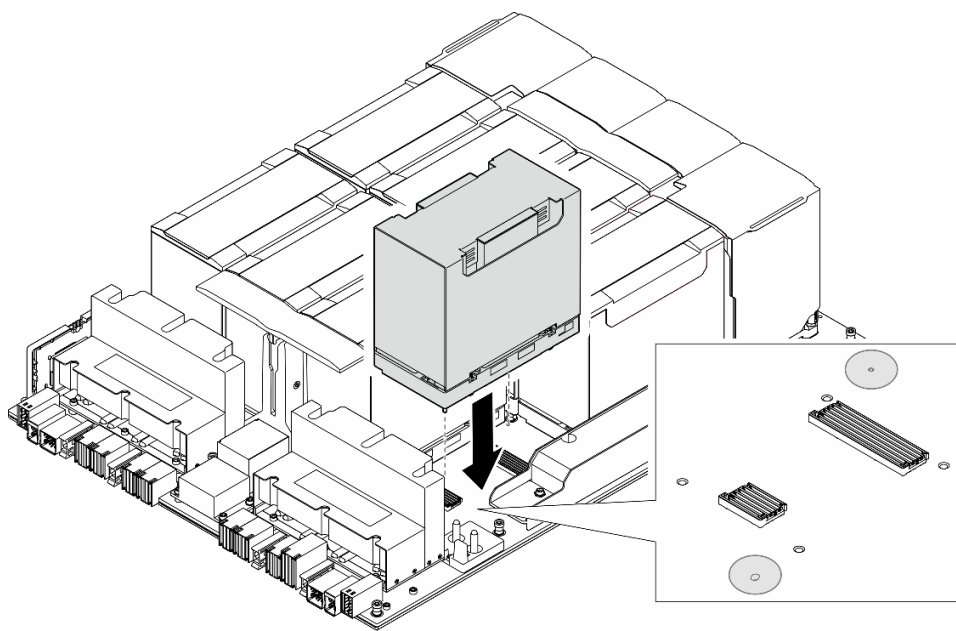
Figura 143. Installazione del Modulo del dissipatore di calore e GPU
