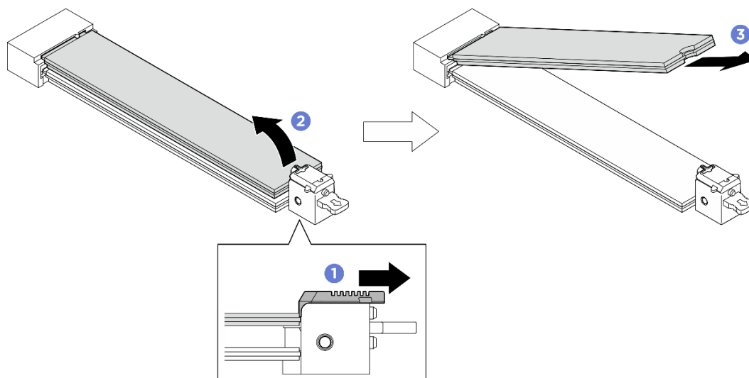
Figura 53. Rimozione dell'unità M.2 superiore
