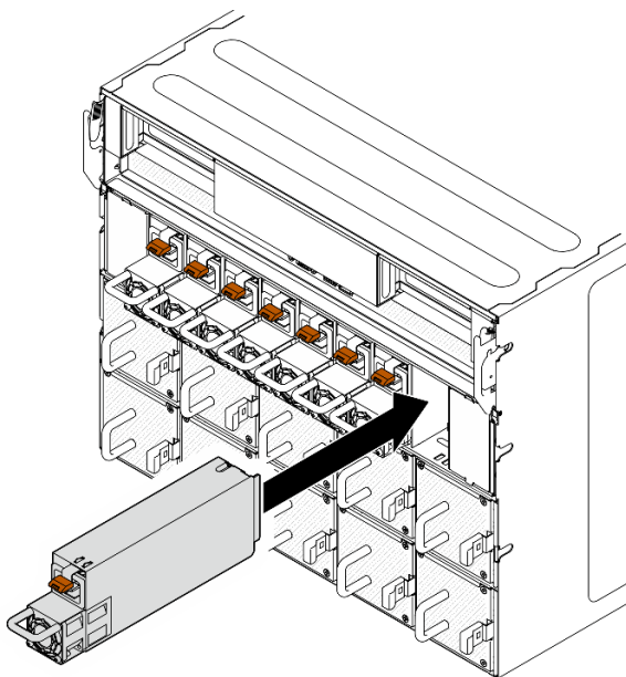
Figura 80. Installazione dell'unità di alimentazione
