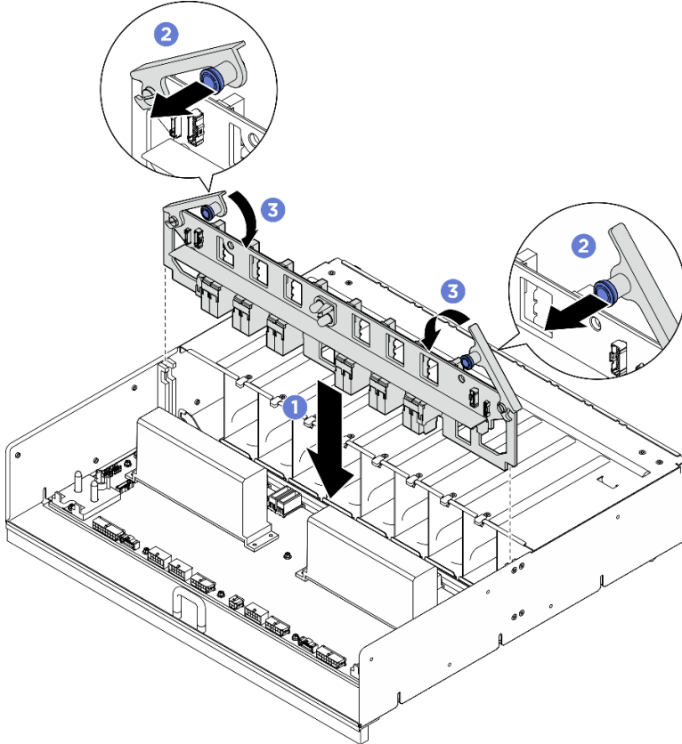
Figura 102. Installazione dell'Interposer PSU
