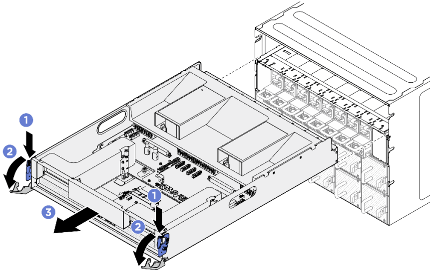
Figura 21. Rimozione dello shuttle di elaborazione 2U
