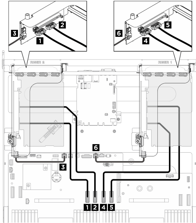
Figura 192. Instradamento dei cavi delle schede verticali PCIe
