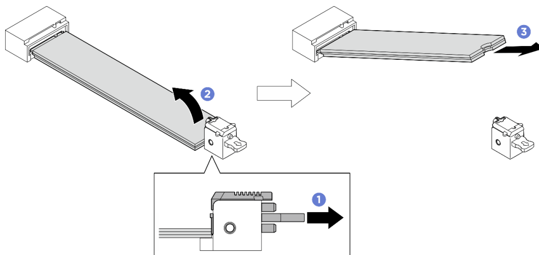
Figura 54. Rimozione dell'unità M.2 inferiore
