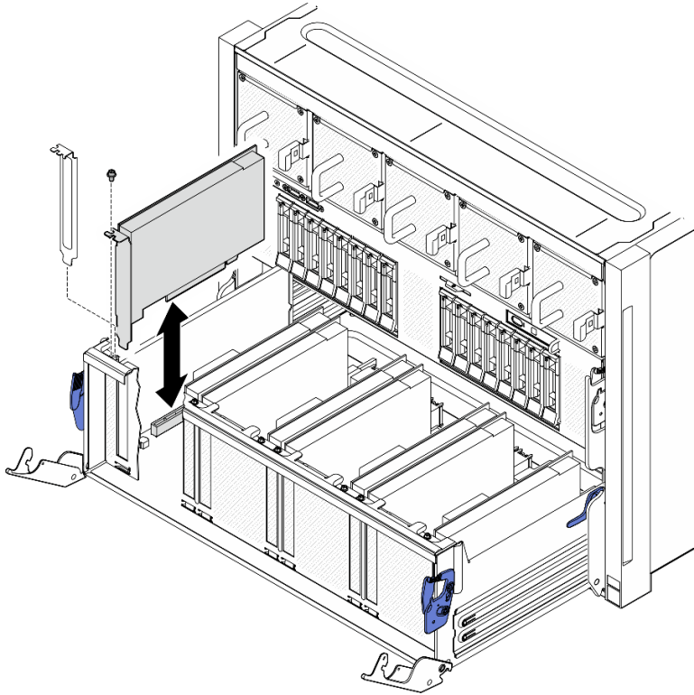
Figura 157. Installazione dell'adattatore PCIe anteriore
