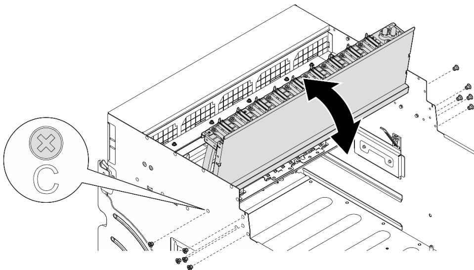
Figura 117. Capovolgimento del cablaggio dello switch PCIe anteriore
