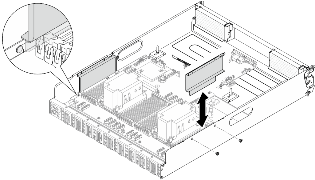
Figura 103. Rimozione della guida del cavo
