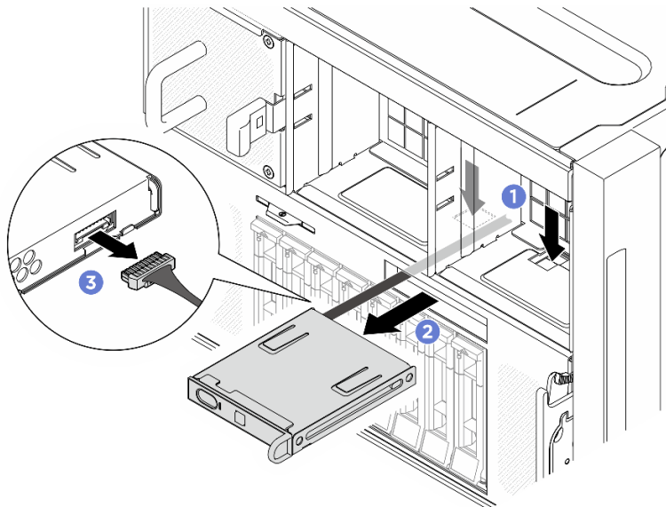
Figura 50. Rimozione del pannello di diagnostica integrato
