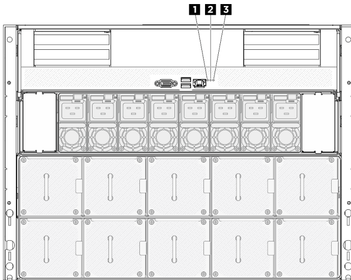
Figura 214. LED di sistema sulla vista posteriore
