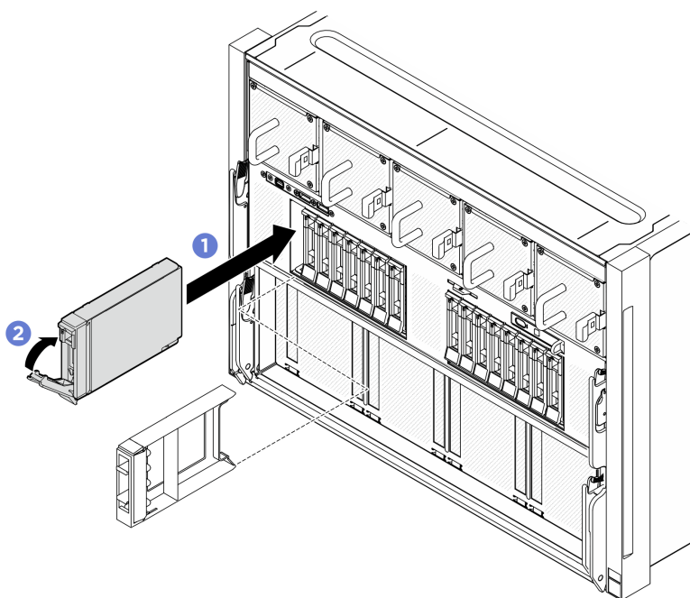
Figura 20. Installazione dell'unità hot-swap da 2,5"
