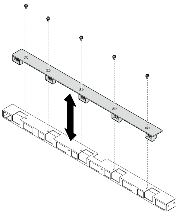
Figura 38. Rimozione scheda di controllo della ventola anteriore
