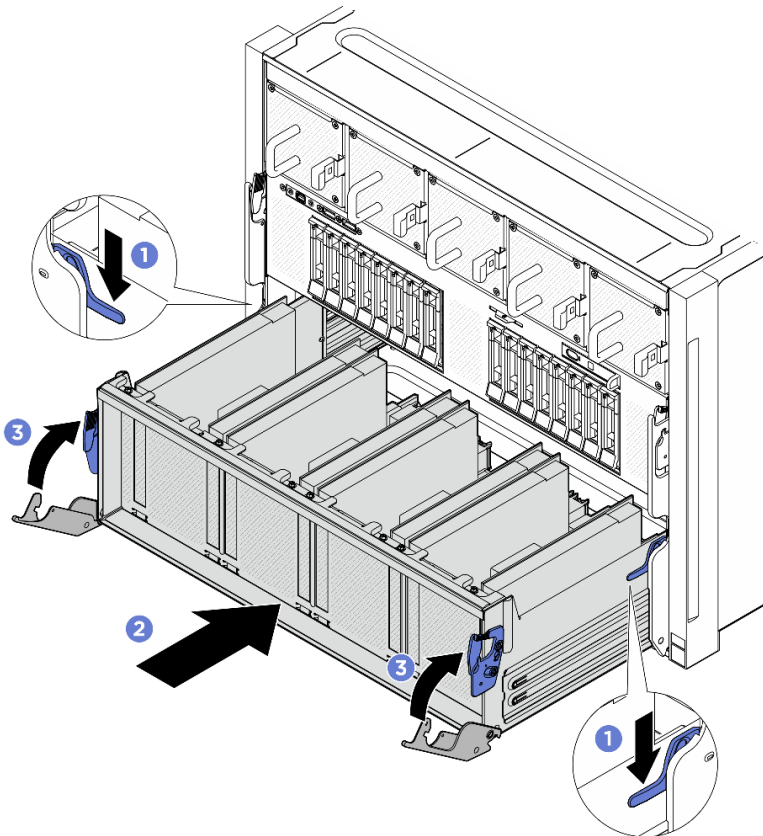
Figura 139. Installazione dello Shuttle dello switch PCIe nello shuttle GPU 8U
