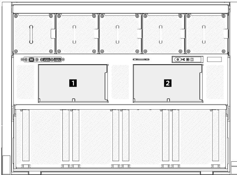
Figura 109. Numerazione dei backplane dell'unità da 2,5"
