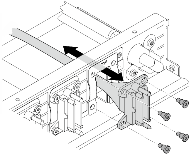
Figura 164. Rimozione del cavo per modulo I/O anteriore, pannello di diagnostica integrato, gestione GPU o segnale
