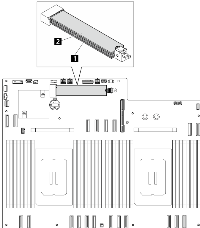
Figura 55. Slot dell'unità M.2
