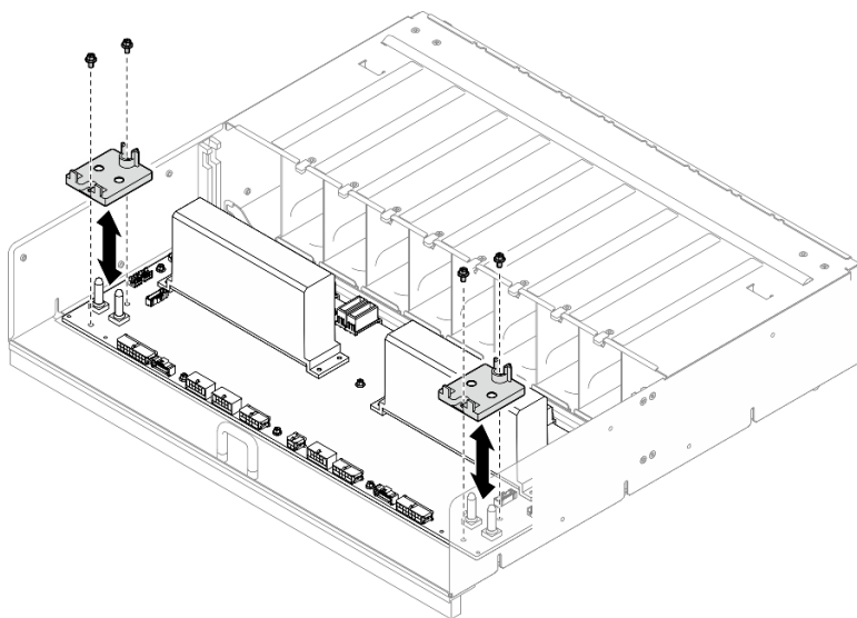
Figura 73. Rimozione fermacavo
