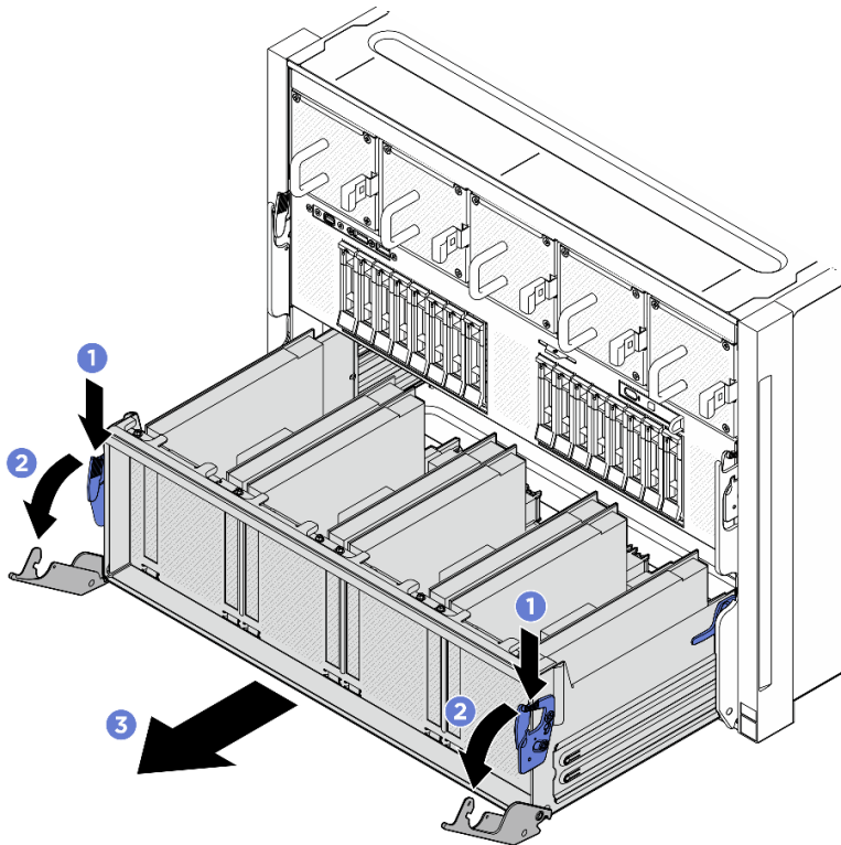
Figura 134. Rimozione dello Shuttle dello switch PCIe in posizione di blocco
