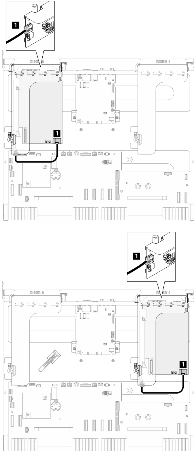
Figura 193. Instradamento dei cavi di alimentazione DPU
