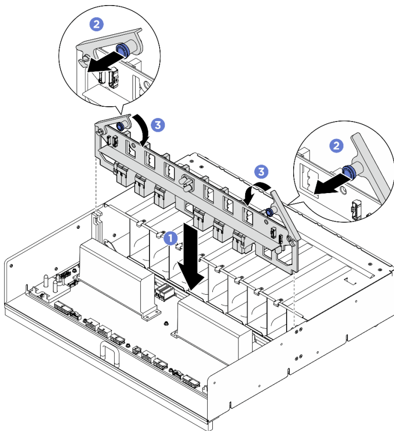
Figura 100. Installazione dell'Interposer PSU
