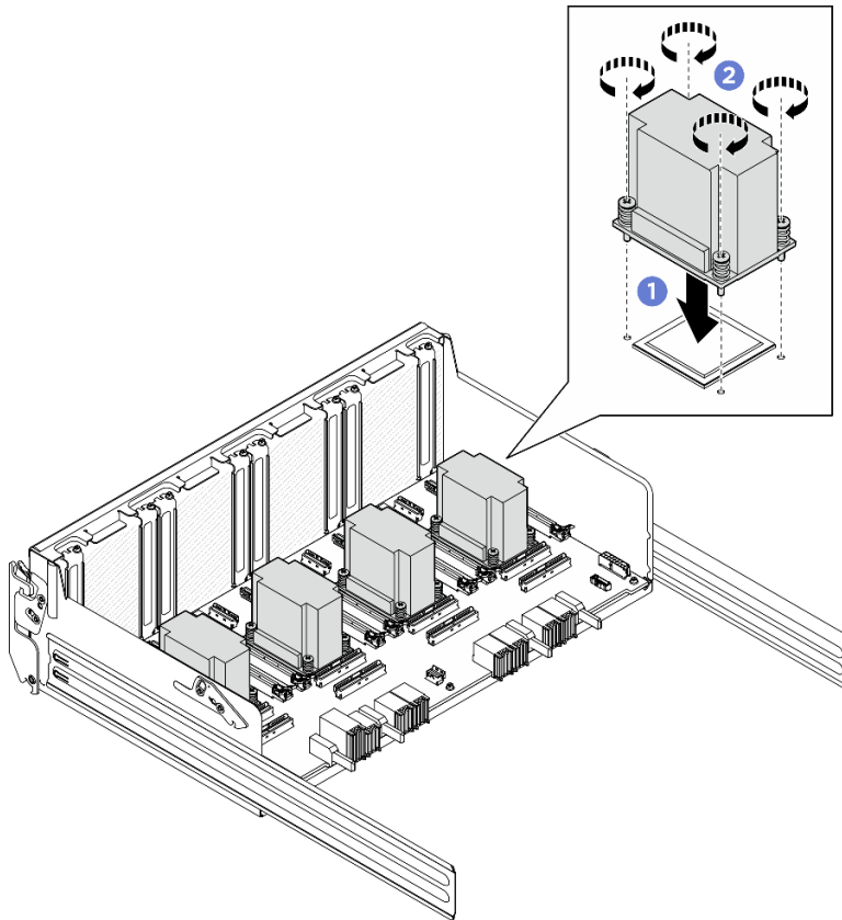
Figura 154. Installazione del Dissipatore di calore della scheda dello switch PCIe
