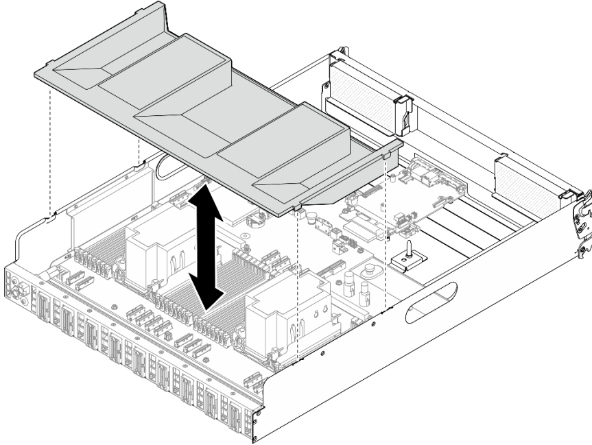
Figura 81. Rimozione del deflettore d'aria del processore
