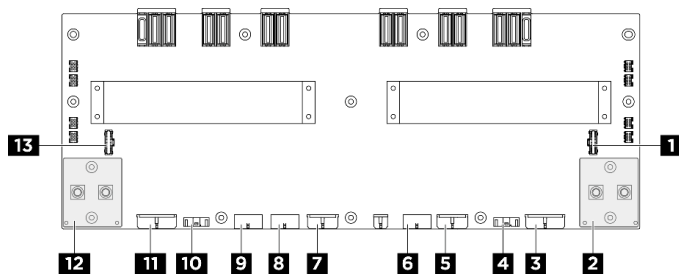
Figura 189. Connettori sulla scheda di distribuzione dell'alimentazione
