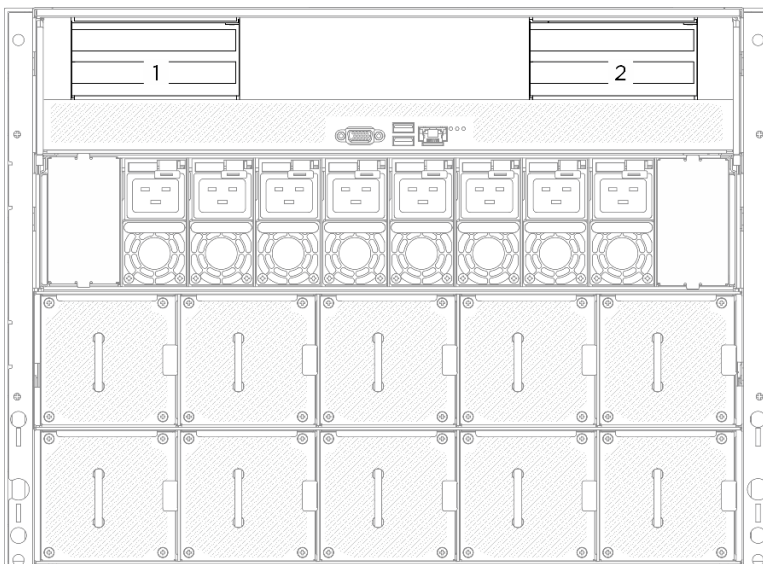
Figura 64. Posizioni schede verticali PCIe
