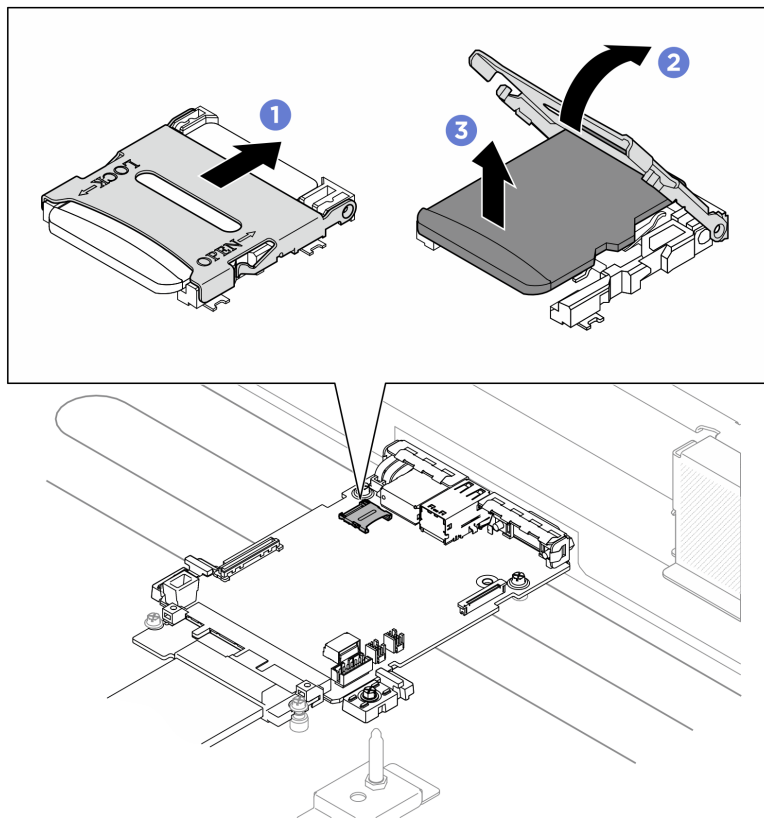
Figura 62. Rimozione della scheda MicroSD
