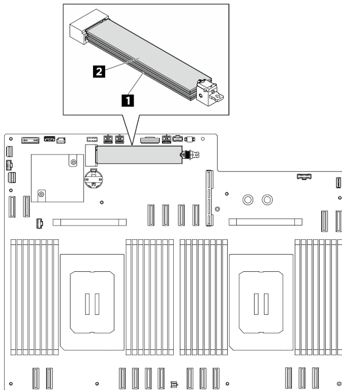
Figura 52. Slot dell'unità M.2
