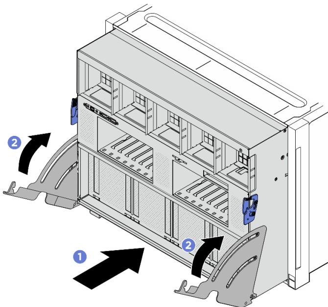
Figura 24. Installazione del shuttle GPU 8U
