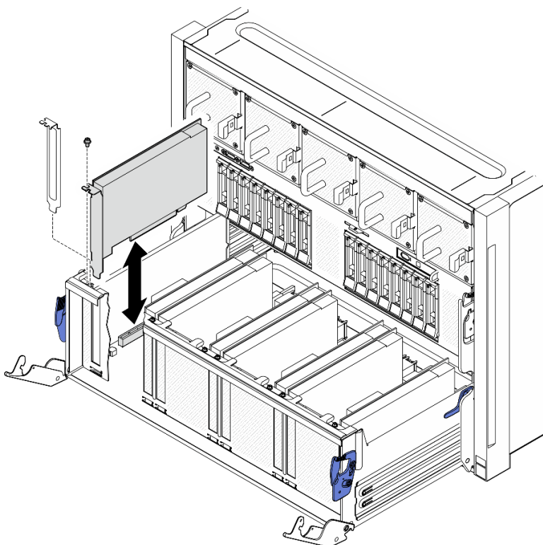
Figura 156. Rimozione dell'adattatore PCIe anteriore
