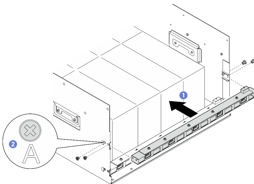
Figura 45. Installazione dell'assieme della scheda di controllo della ventola posteriore
