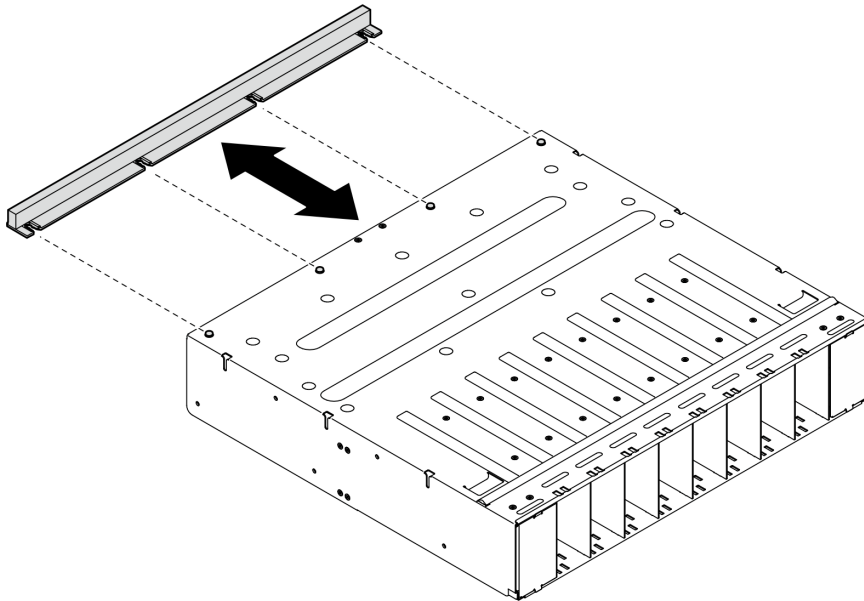
Figura 48. Rimozione del deflettore d'aria GPU
