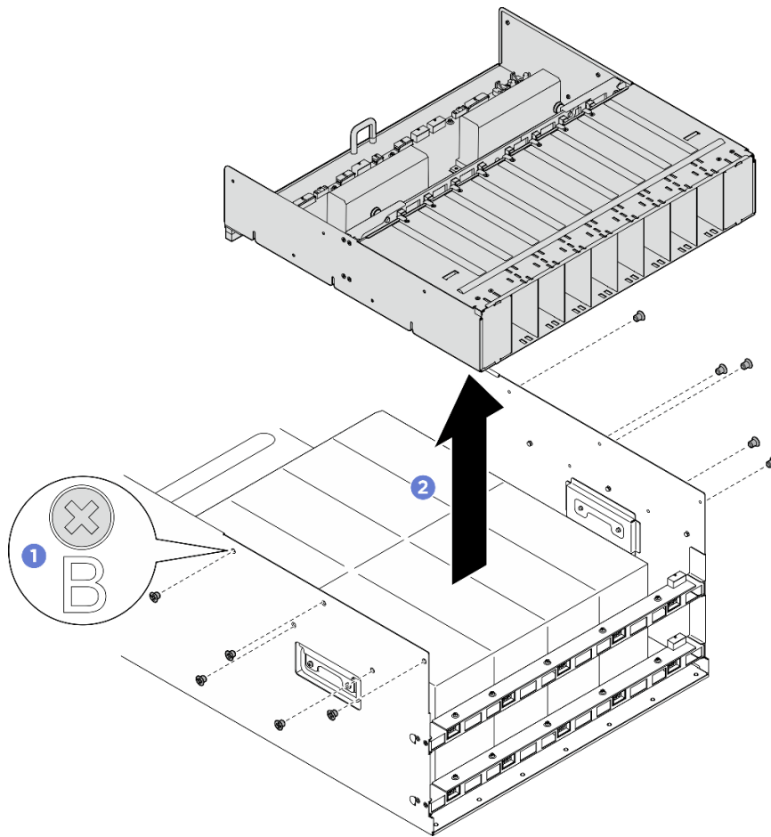
Figura 71. Rimozione del Complesso di alimentazione
