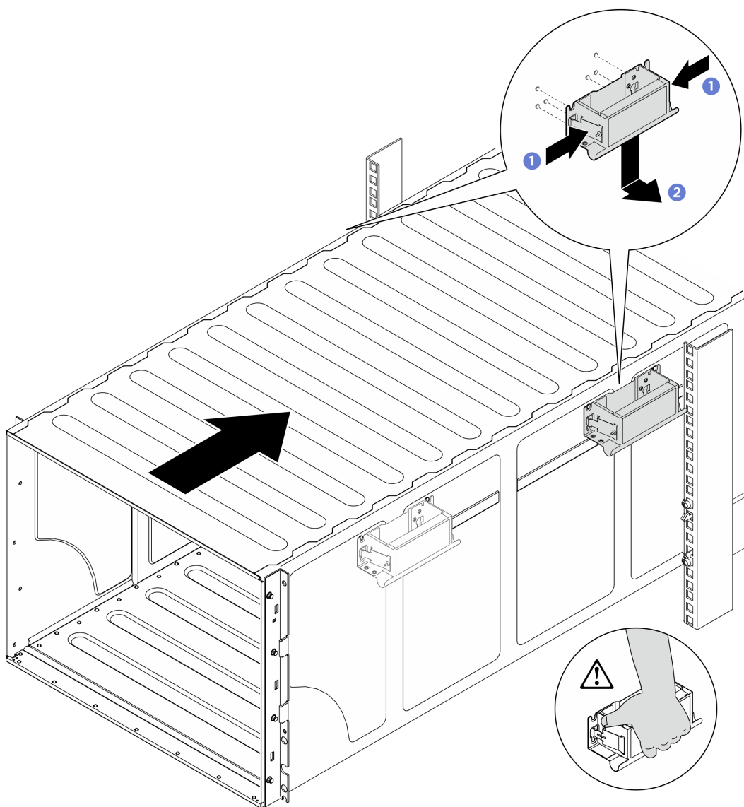
Figura 11. Rimozione della maniglia posteriore
