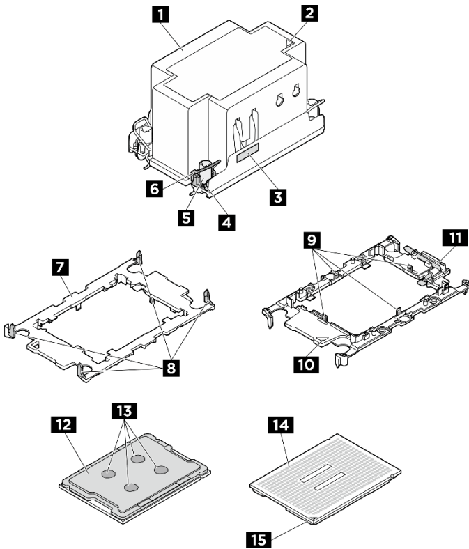
Figura 85. Componenti del PHM
