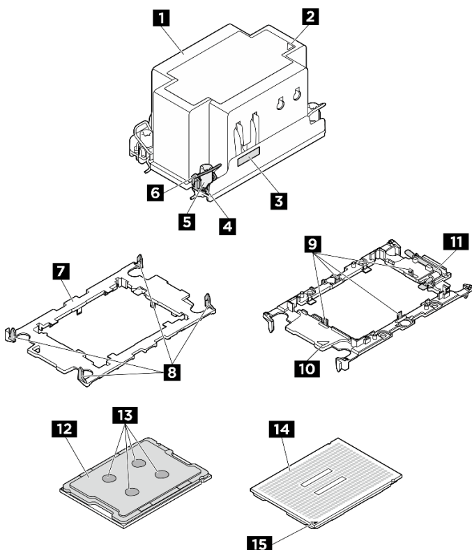
Figura 86. Componenti del PHM
