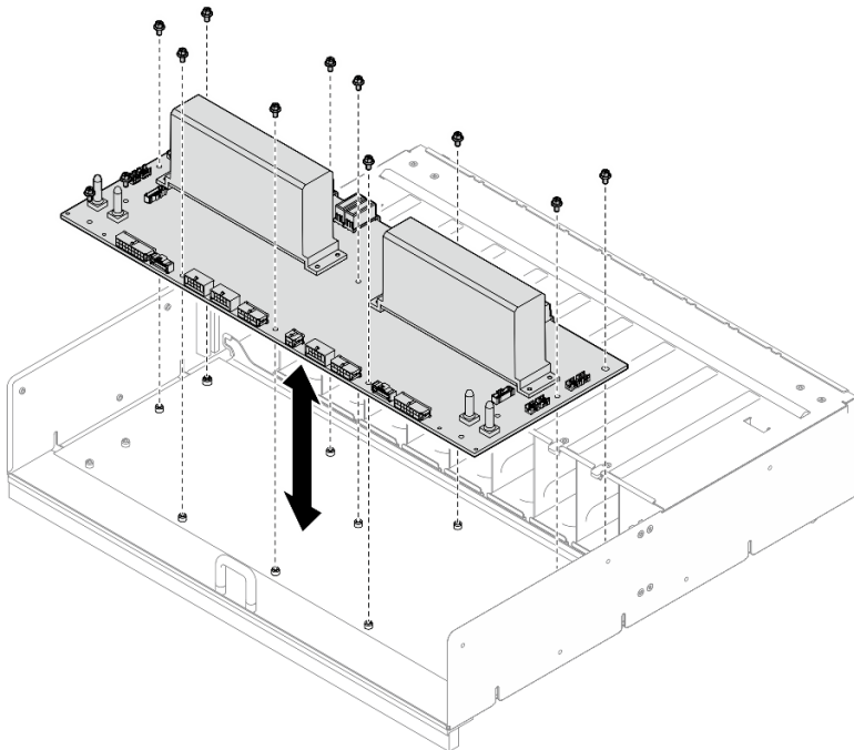
Figura 75. Installazione della scheda di distribuzione dell'alimentazione
