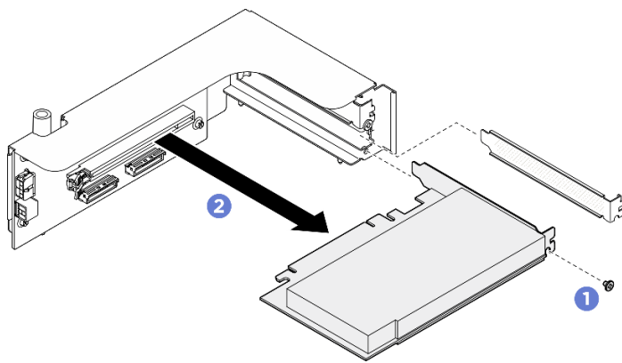
Figura 66. Rimozione dell'adattatore PCIe posteriore
