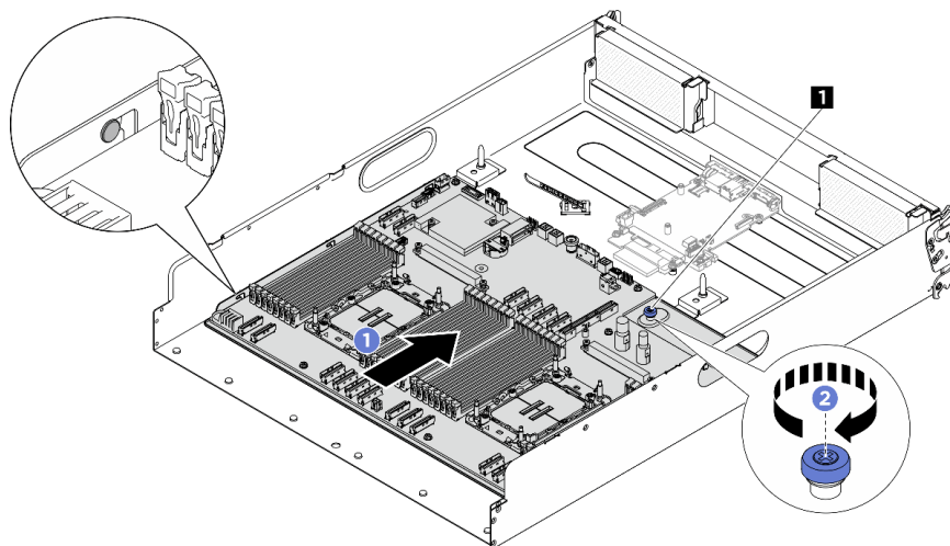
Figura 107. Fissaggio della scheda di sistema
