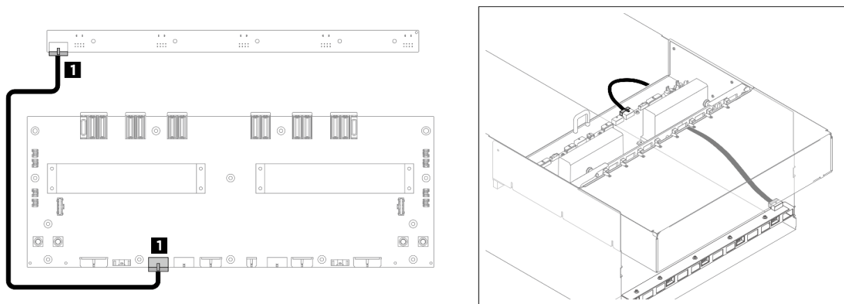
Figura 196. Instradamento dei cavi sulla scheda di controllo della ventola posteriore (inferiore)
