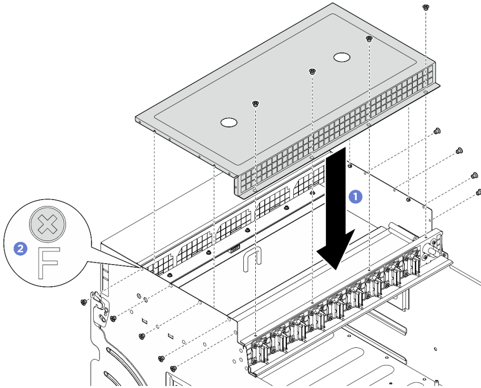
Figura 26. Installazione del pannello di copertura del cavo
