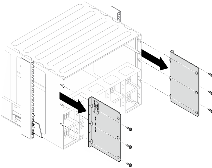
Figura 2. Rimozione della staffa di supporto superiore
