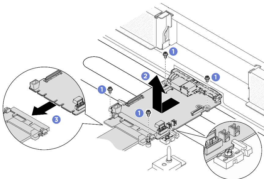
Figura 83. Rimozione della scheda I/O di sistema
