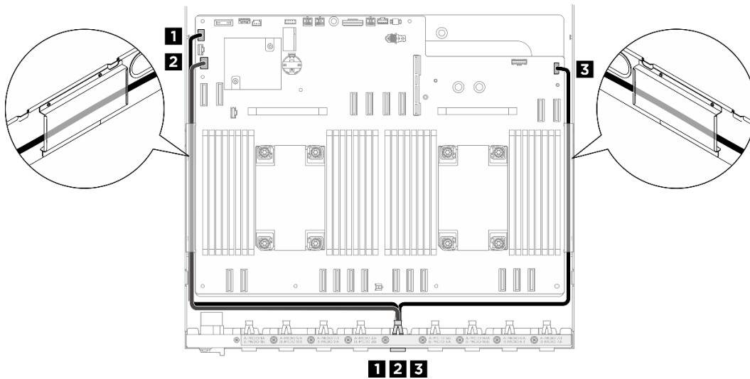
Figura 197. Instradamento dei cavi del modulo I/O anteriore e del pannello di diagnostica integrato
