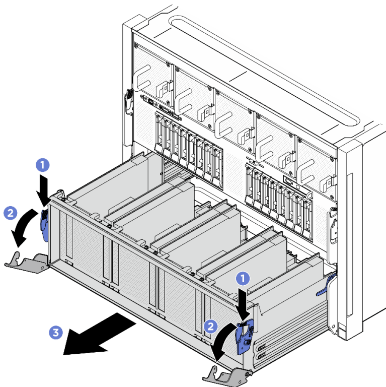
Figura 125. Rimozione dello Shuttle dello switch PCIe in posizione di blocco
