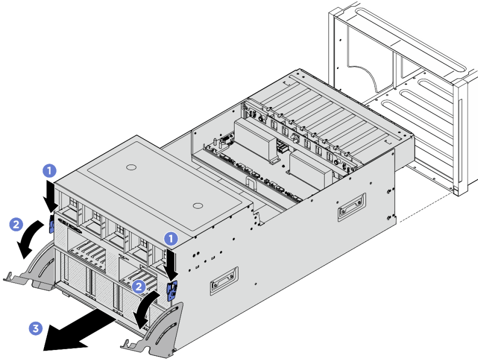
Figura 23. Rimozione del shuttle GPU 8U
