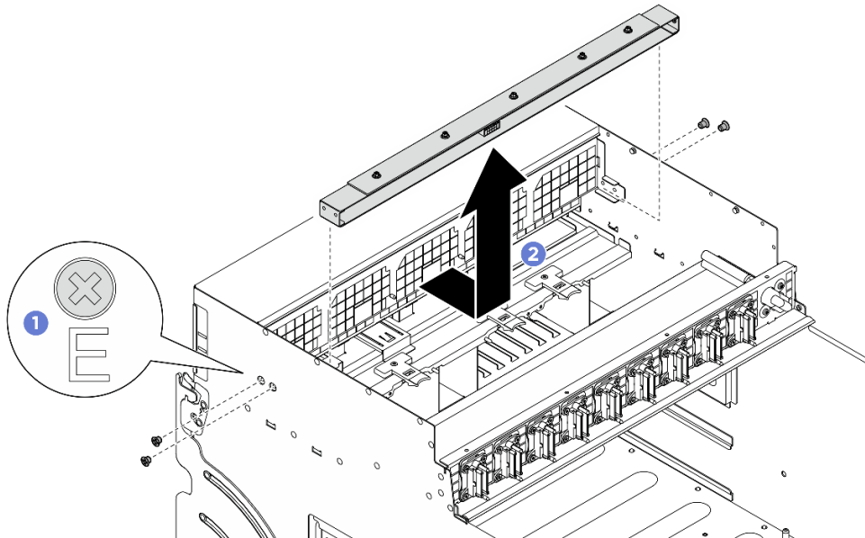
Figura 37. Rimozione dell'insieme della scheda di controllo della ventola anteriore
