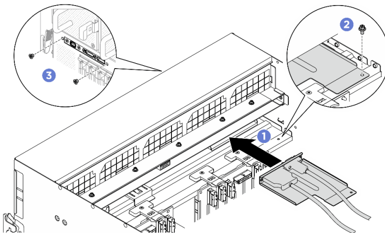
Figura 171. Installazione del modulo I/O anteriore
