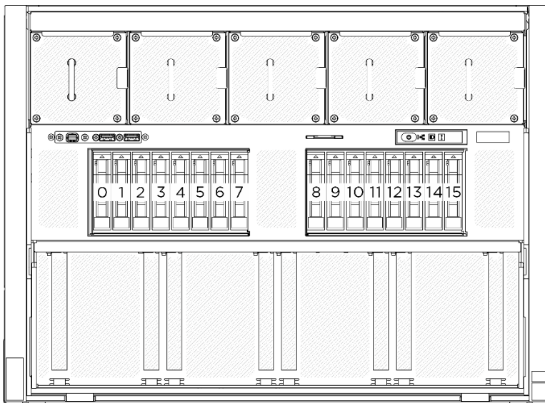
Figura 17. Numerazione del vano dell'unità da 2,5"
