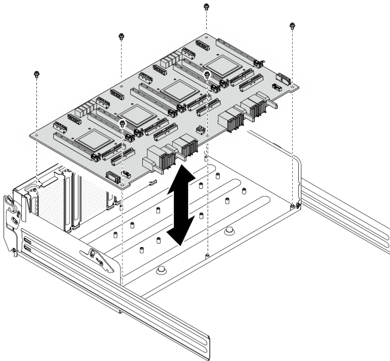
Figura 151. Rimozione del Scheda dello switch PCIe
