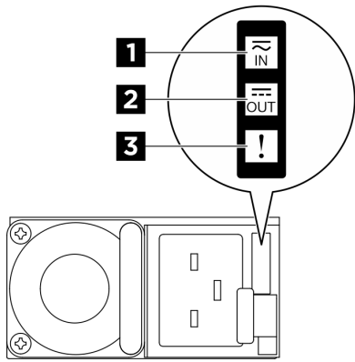
Figura 213. LED dell'alimentatore CFFv4
