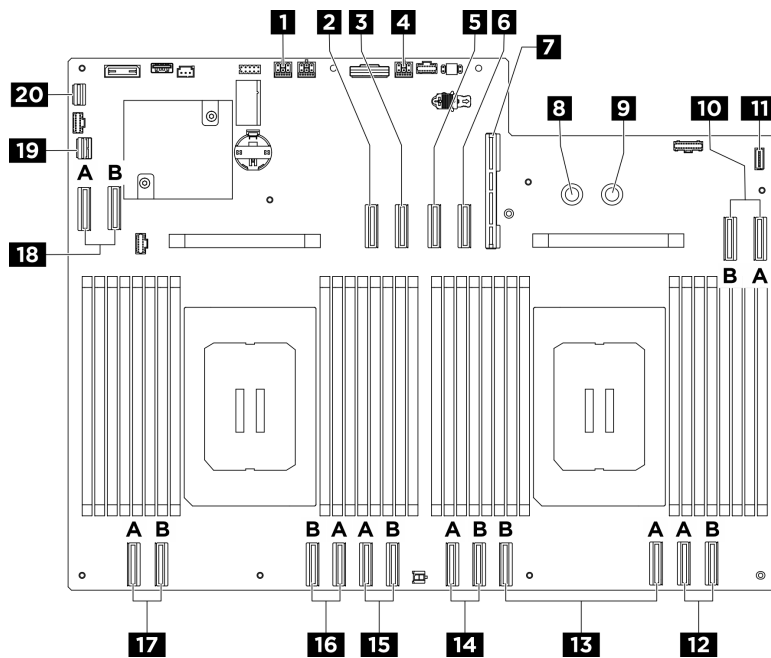
Figura 191. Connettori della scheda di sistema per l'instradamento dei cavi
