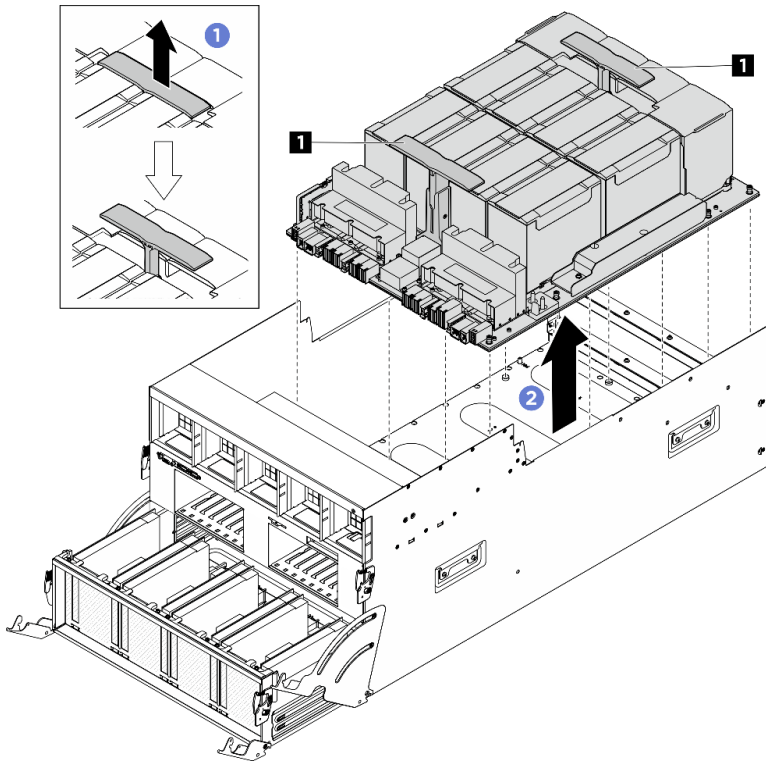
Figura 128. Rimozione del Complesso GPU
