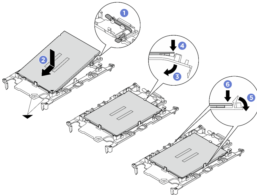
Figura 91. Installazione di una piastra del processore
