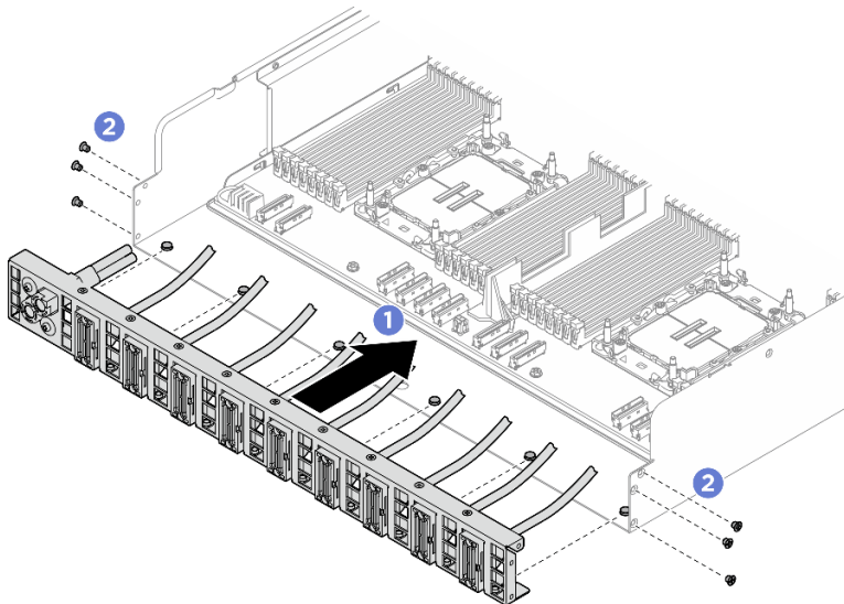
Figura 177. Installazione del Cablaggio dello switch PCIe posteriore
