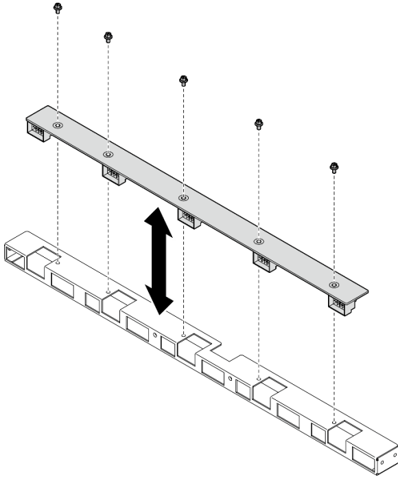
Figura 43. Rimozione della scheda di controllo della ventola posteriore
