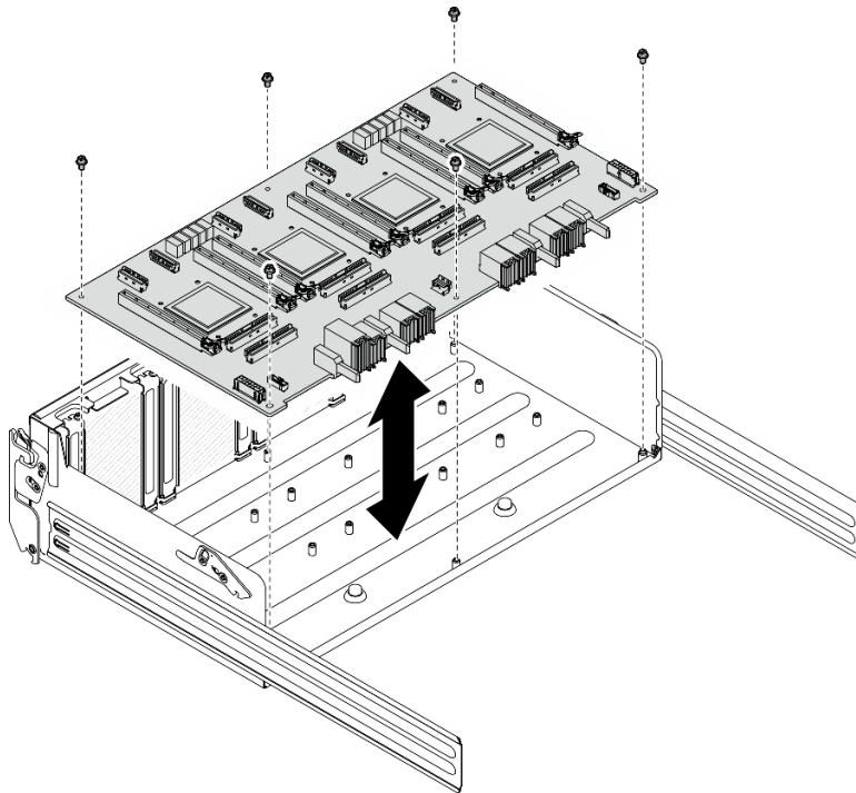
Figura 152. Installazione della Scheda dello switch PCIe
