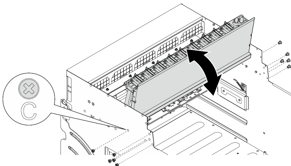
Figura 138. Capovolgimento del cablaggio dello switch PCIe anteriore
