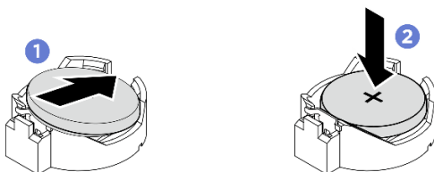
Figura 30. Installazione della batteria CMOS
