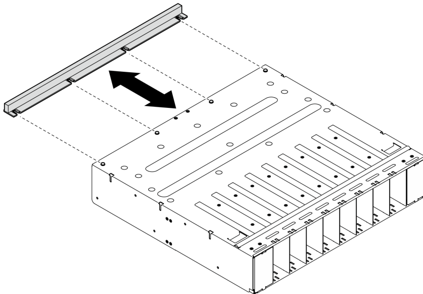
Figura 49. Installazione del deflettore d'aria GPU
