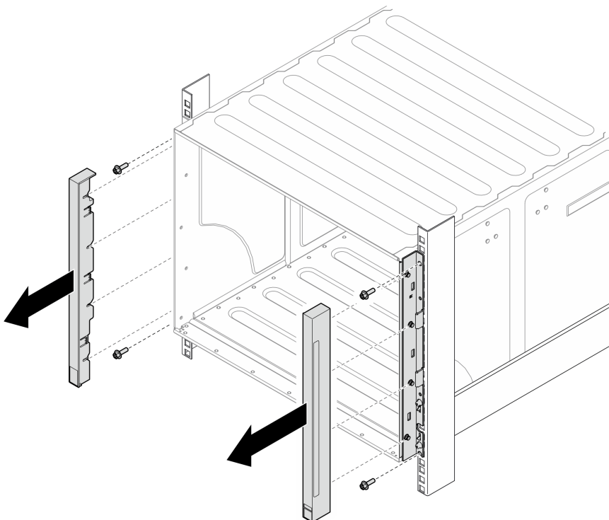
Figura 4. Rimozione del coperchio EIA
