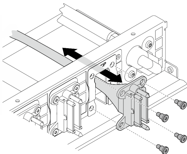
Figura 167. Installazione del cavo per modulo I/O anteriore, pannello di diagnostica integrato, gestione GPU o segnale
