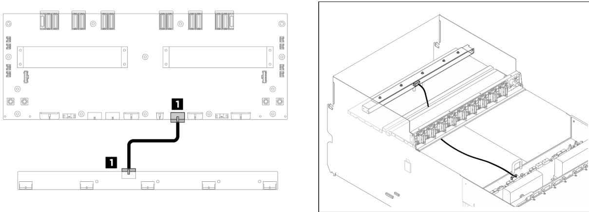
Figura 194. Instradamento dei cavi della scheda di controllo della ventola anteriore
