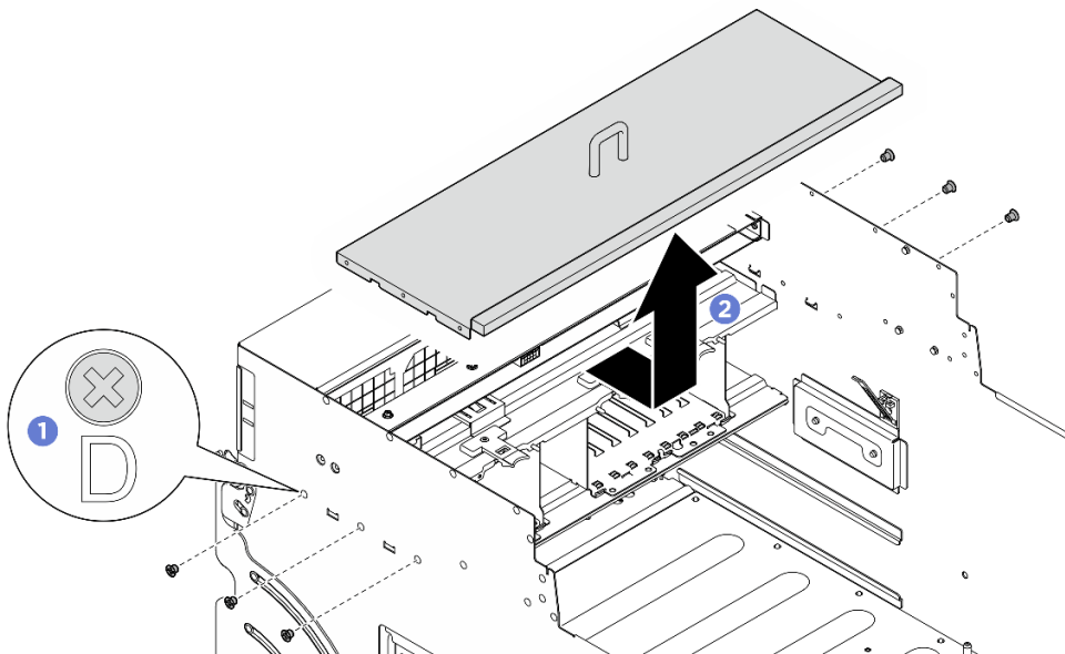
Figura 148. Rimozione del coperchio I/O
