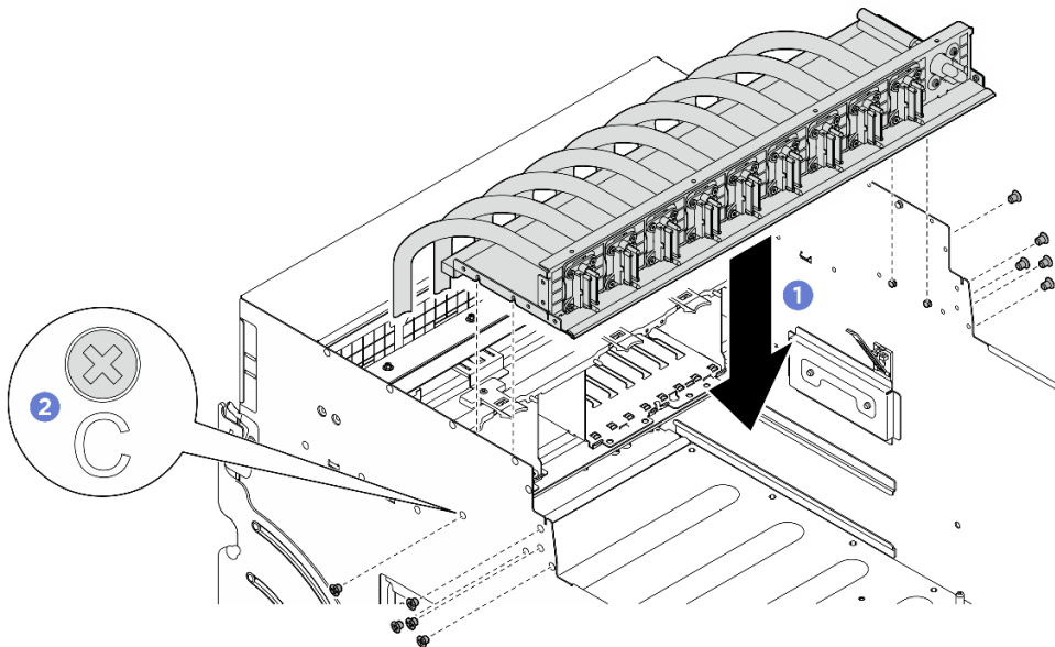
Figura 169. Installazione del Cablaggio dello switch PCIe anteriore
