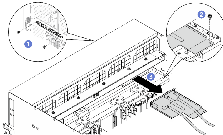
Figura 161. Rimozione del modulo I/O anteriore
