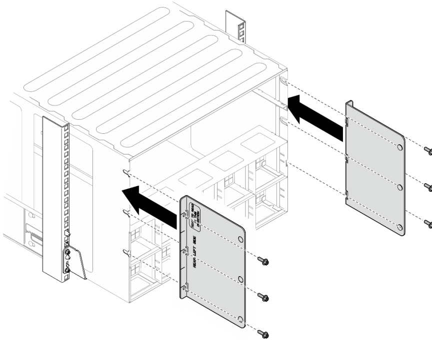
Figura 16. Installazione della staffa di supporto superiore
