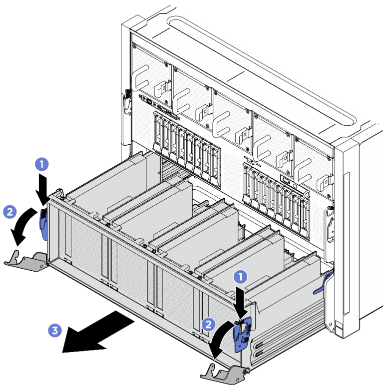
Figura 178. Rimozione dello Shuttle dello switch PCIe in posizione di blocco
