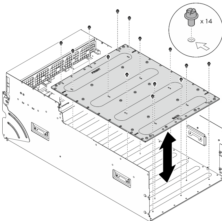
Figura 137. Installazione della Piastra adattatore del complesso GPU
