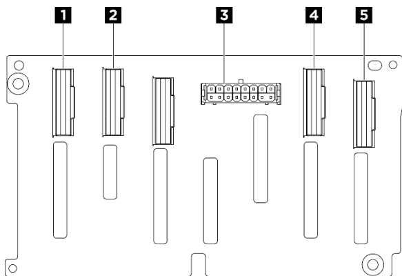
Figura 182. Connettori del backplane NVMe da 2,5 pollici
