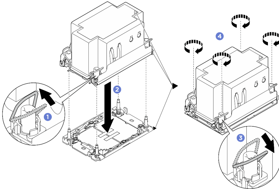
Figura 94. Installazione del PHM
