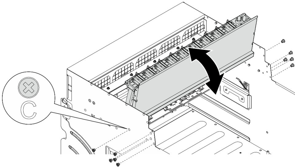
Figura 126. Capovolgimento del cablaggio dello switch PCIe anteriore
