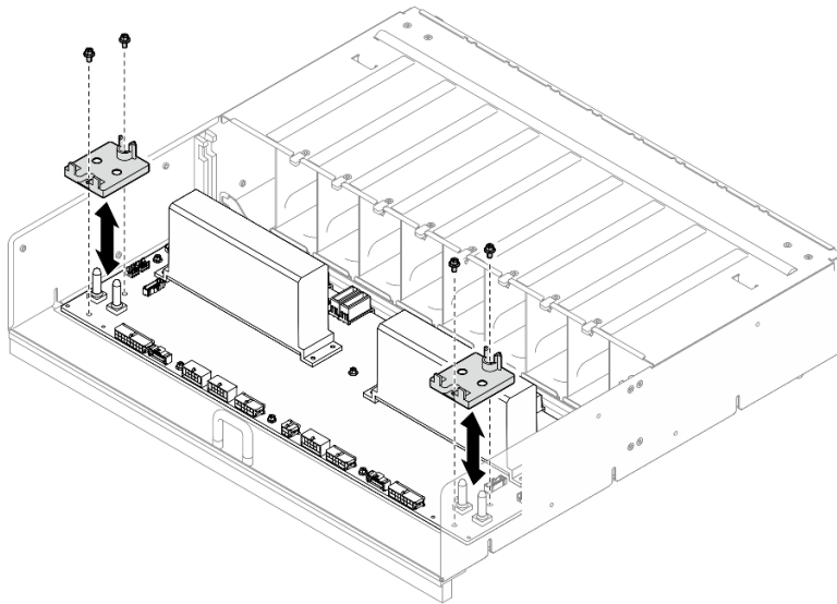
Figura 99. Installazione del fermacavo
