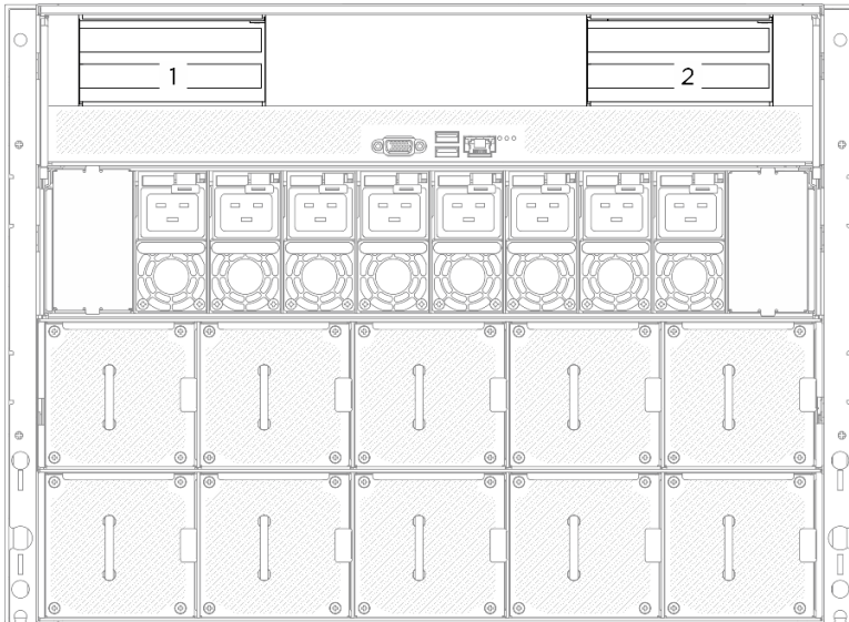
Figura 68. Posizioni schede verticali PCIe
