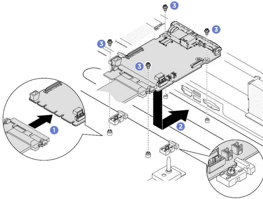
Figura 84. Installazione della scheda I/O di sistema
