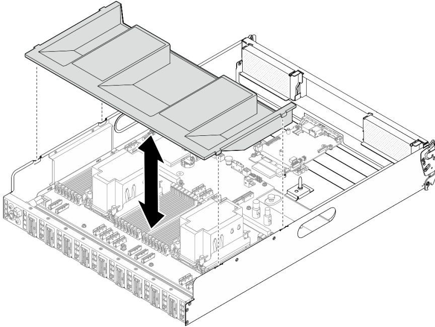
Figura 82. Installazione del deflettore d'aria del processore
