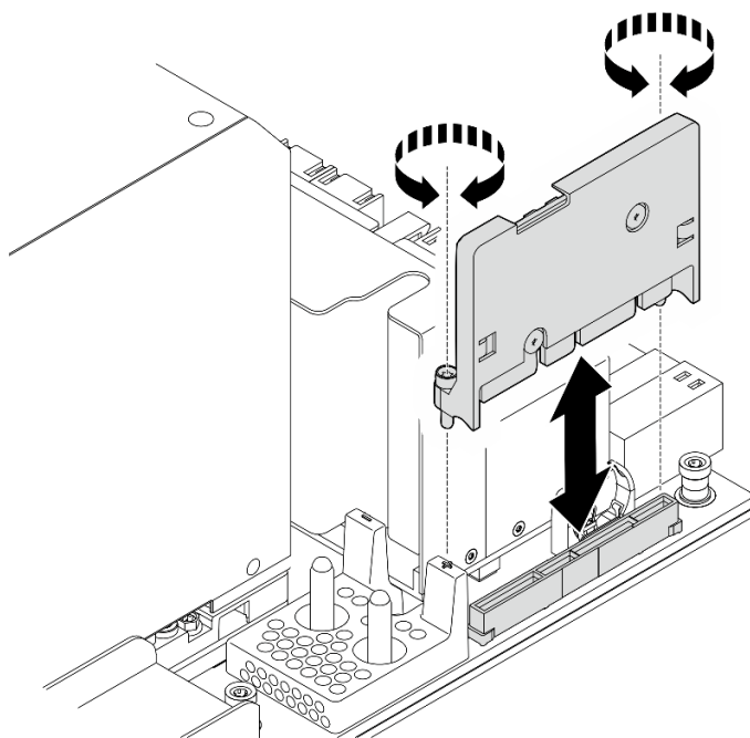
Figura 147. Installazione della scheda HMC
