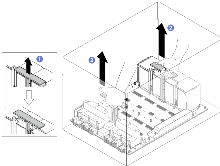
Figura 120. Rimozione della Scheda di base GPU dalla confezione
