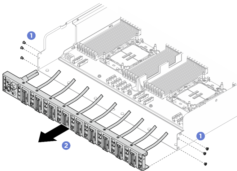
Figura 172. Rimozione del Cablaggio dello switch PCIe posteriore
