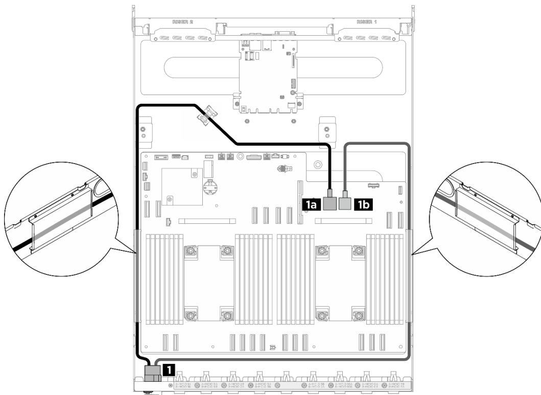
Figura 200. Instradamento dei cavi di alimentazione per i cavi di alimentazione
