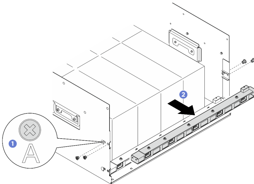
Figura 42. Rimozione dell'assieme della scheda di controllo della ventola posteriore
