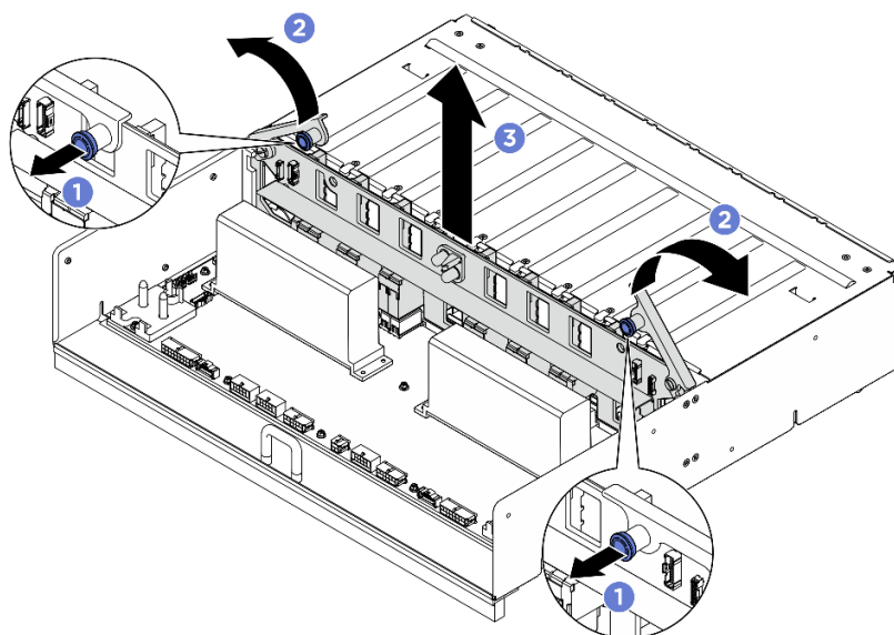
Figura 101. Rimozione del Interposer PSU
