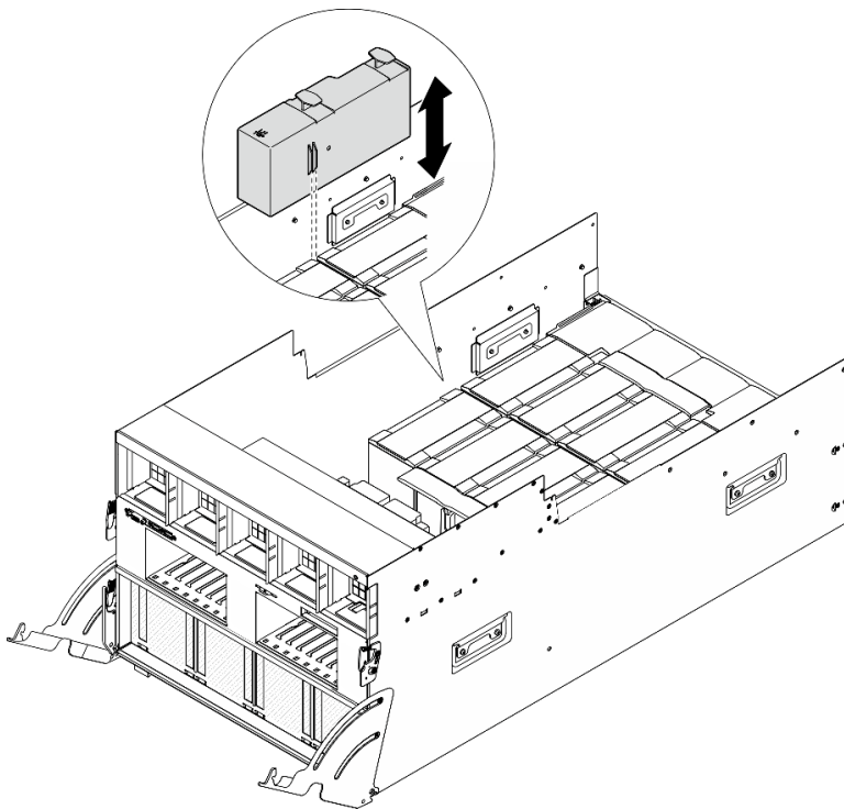
Figura 114. Rimozione del condotto dell'aria GPU
