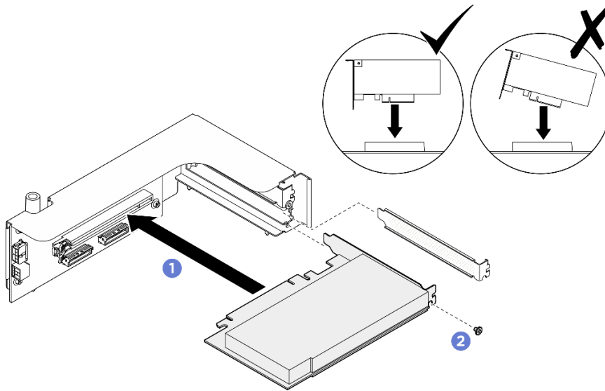
Figura 160. Installazione dell'adattatore PCIe posteriore
