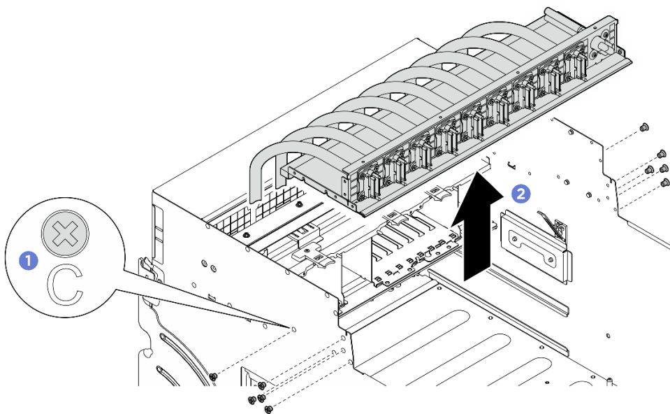
Figura 163. Rimozione del Cablaggio dello switch PCIe anteriore
