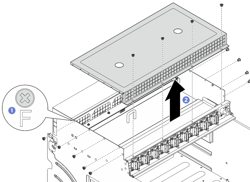
Figura 25. Rimozione del pannello di copertura del cavo
