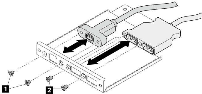
Figura 170. Installazione dei cavi del modulo I/O anteriore
