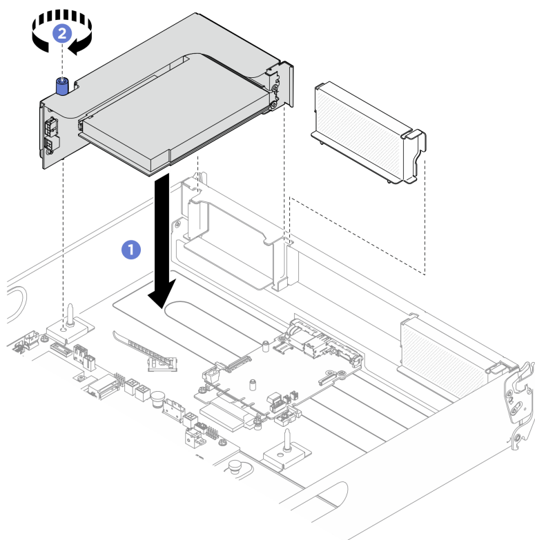
Figura 70. Installazione dell'assieme verticale PCIe
