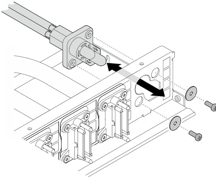
Figura 165. Rimozione del cavo di alimentazione
