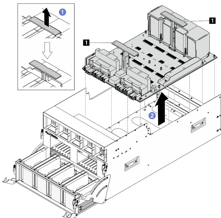
Figura 119. Rimozione del Scheda di base GPU
