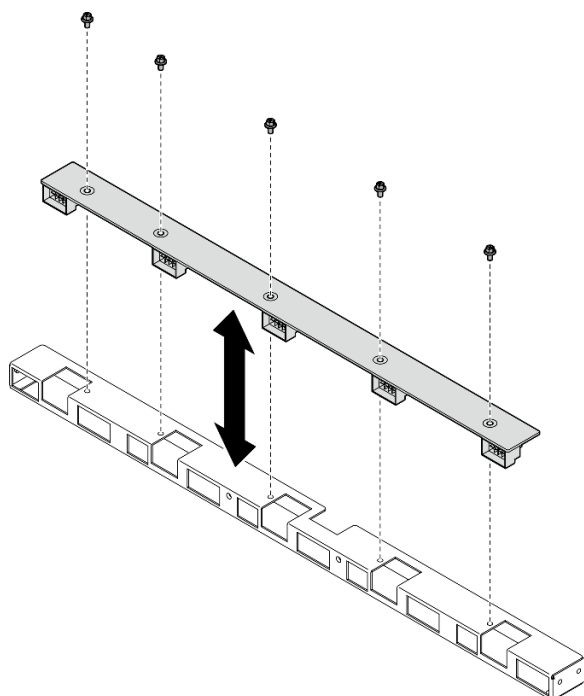
Figura 39. Installazione della scheda di controllo della ventola anteriore
