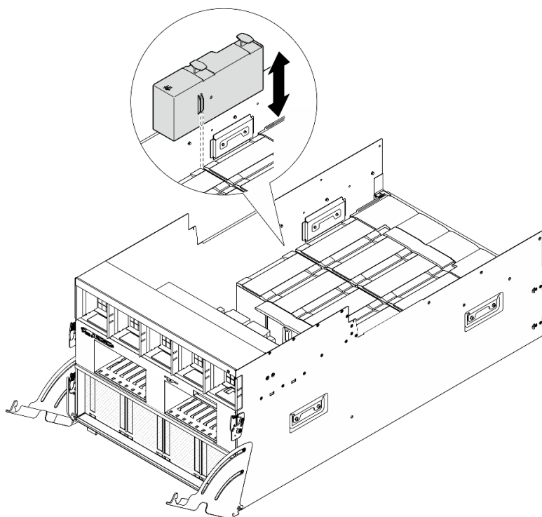
Figura 115. Installazione del condotto dell'aria GPU
