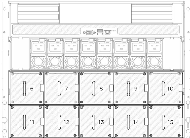
Figura 35. Numerazione delle ventole posteriori
