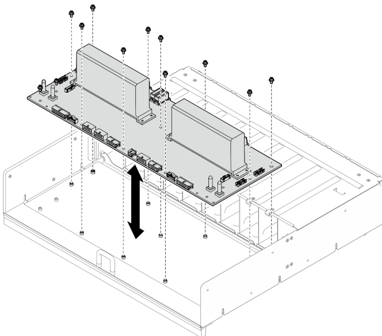
Figura 97. Rimozione della scheda di distribuzione dell'alimentazione
