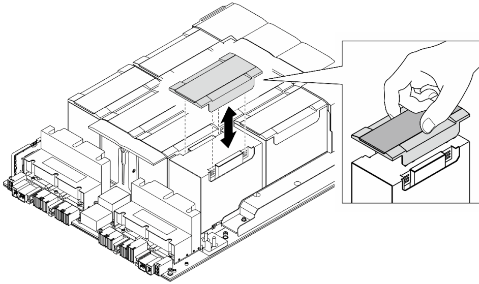
Figura 145. Installazione del coperchio in plastica
