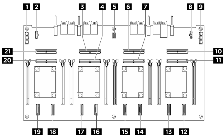
Figura 186. Connettori sulla Scheda dello switch PCIe
