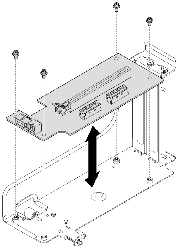
Figura 67. Rimozione della scheda verticale PCIe
