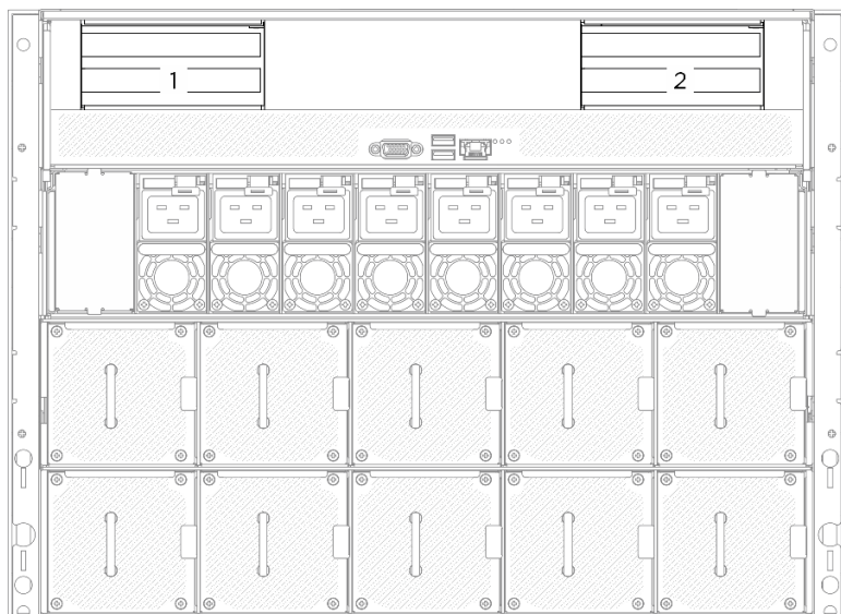
図 68. PCIe ライザーの位置
