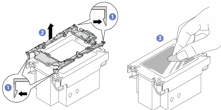
図 89. ヒートシンクからプロセッサ・キャリアを取り外す
