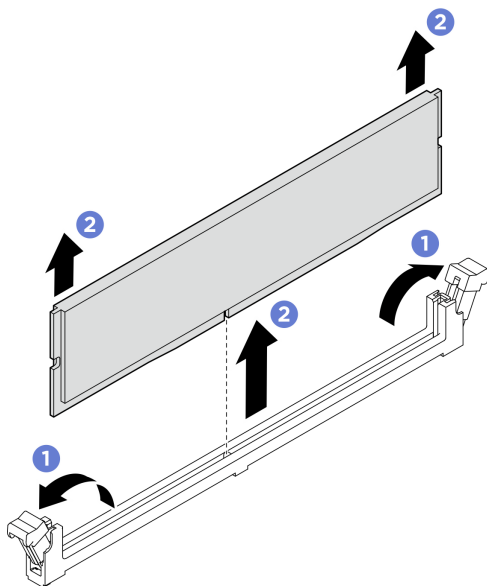
図59. メモリー・モジュールの取り外し
