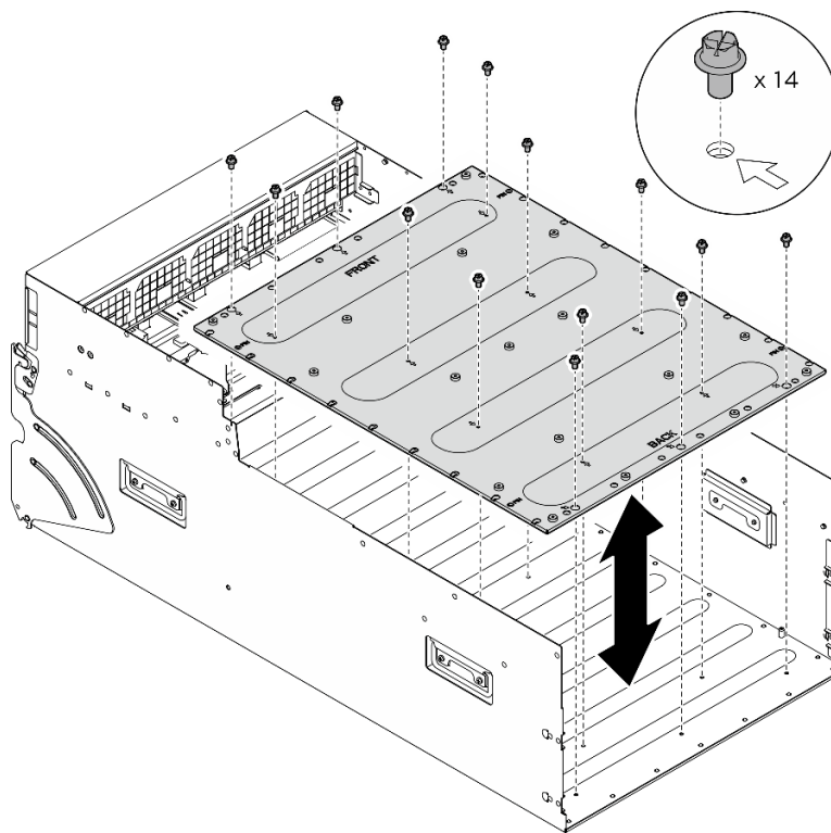
図 137. GPU 複合システム・アダプター・プレートの取り付け
