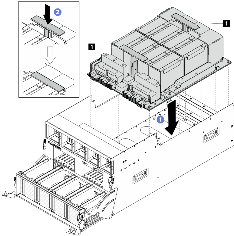
図 130. GPU 複合システムの取り付け
