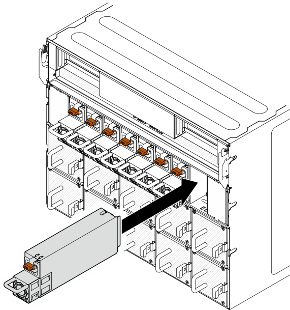
図 80. パワー・サプライ・ユニットの取り付け
