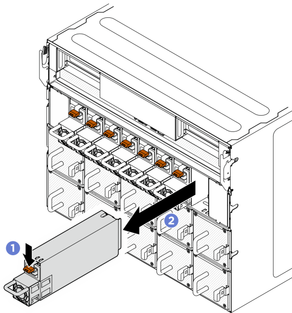
図78. パワー・サプライ・ユニットの取り外し
