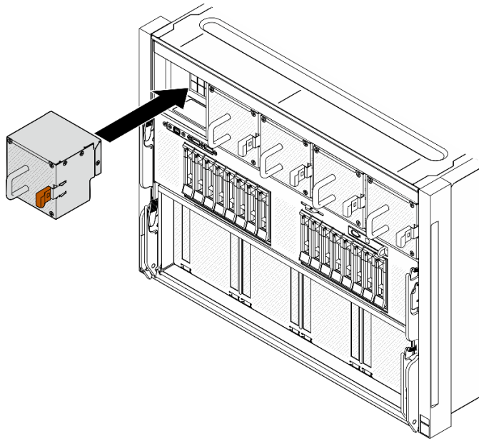
図36. ホット・スワップ・ファンの取り付け
