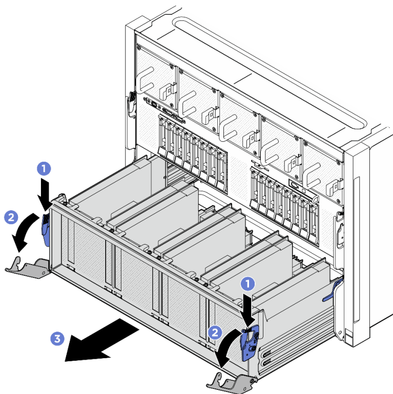
図 155. 停止位置までの PCIe スイッチ・シャトルの取り外し
