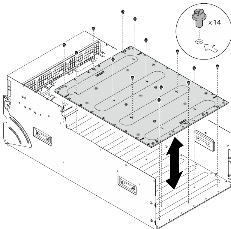
図 136. GPU 複合システム・アダプター・プレートの取り外し
