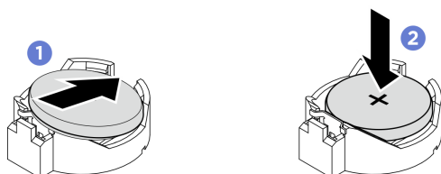
図30. CMOS バッテリーの取り付け
