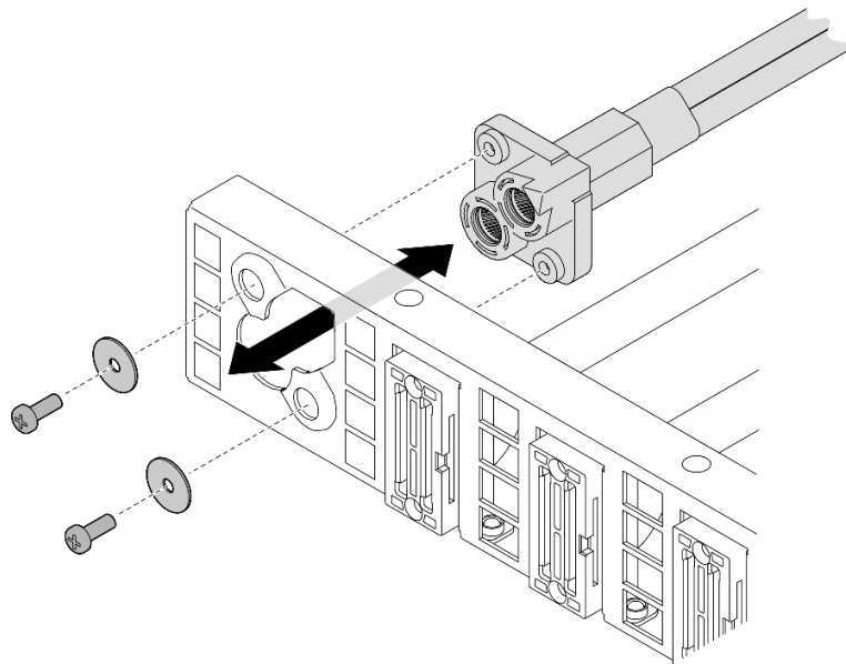
図 176. 電源ケーブルの取り付け
