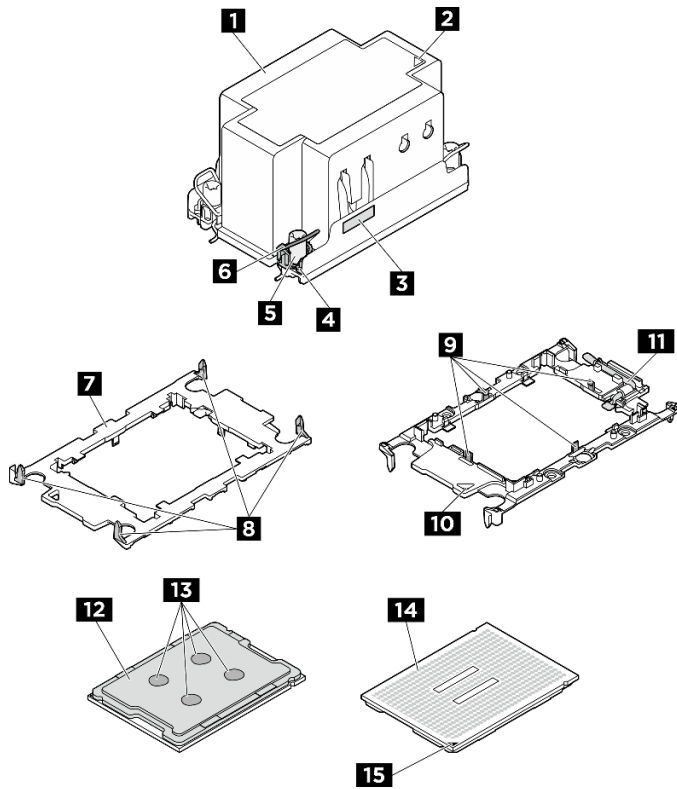
図90. PHM コンポーネント
