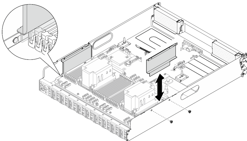
図 103. ケーブル・ガイドの取り外し
