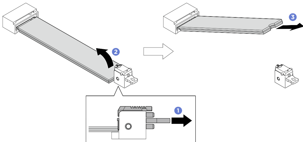
図 54. 下段の M.2 ドライブの取り外し
