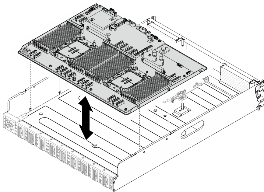
図105. システム・ボードの取り外し
