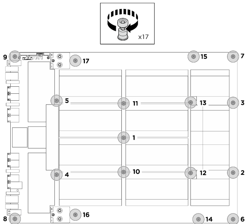
図 122. ねじの取り付け
