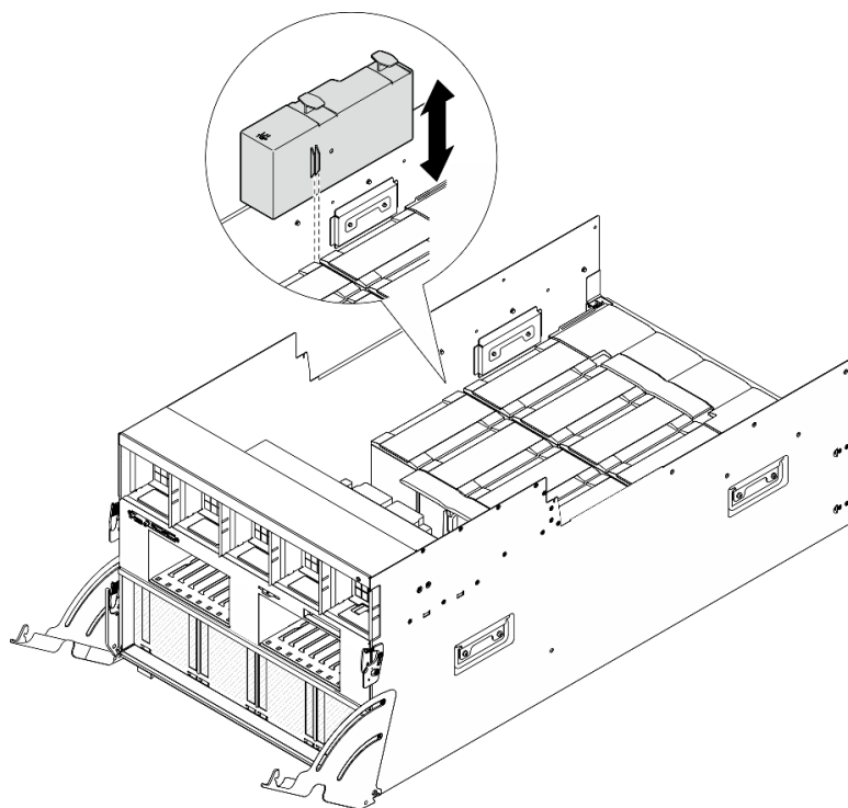
図 115. GPU エアー・ダクトの取り付け
