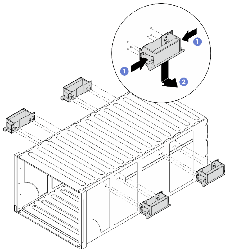
図8. ハンドルの取り外し
