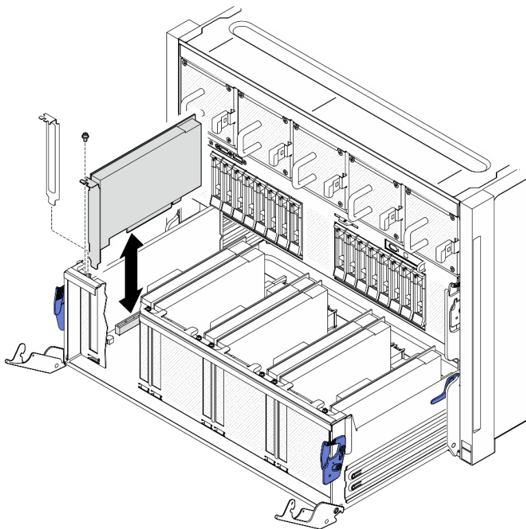
図 157. 前面 PCIe アダプターの取り付け
