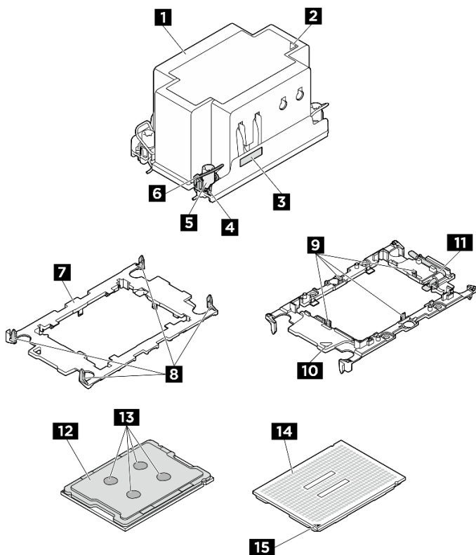
図 85. PHM コンポーネント
