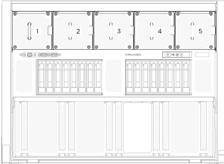
図 34. 前面ファン番号
