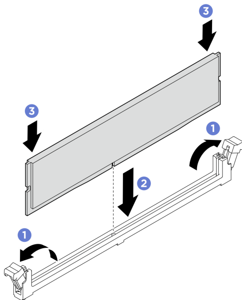
図 61. メモリー・モジュールの取り付け
