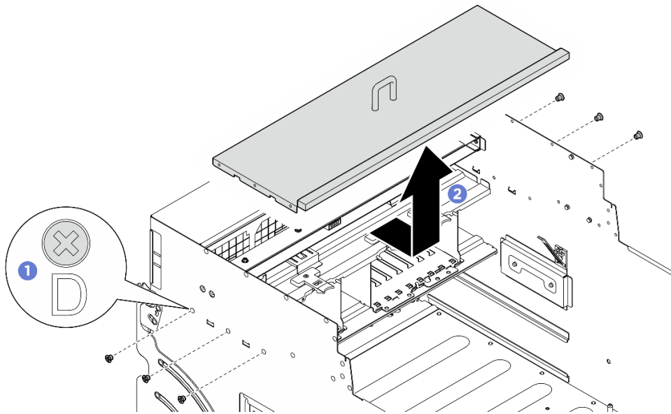
図148. I/O カバーの取り外し
