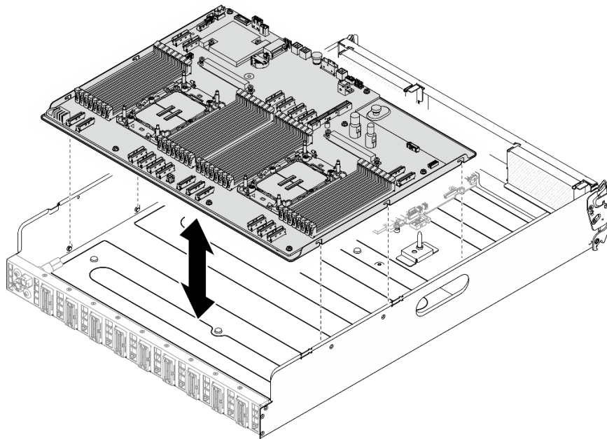
図106. システム・ボードの取り付け
