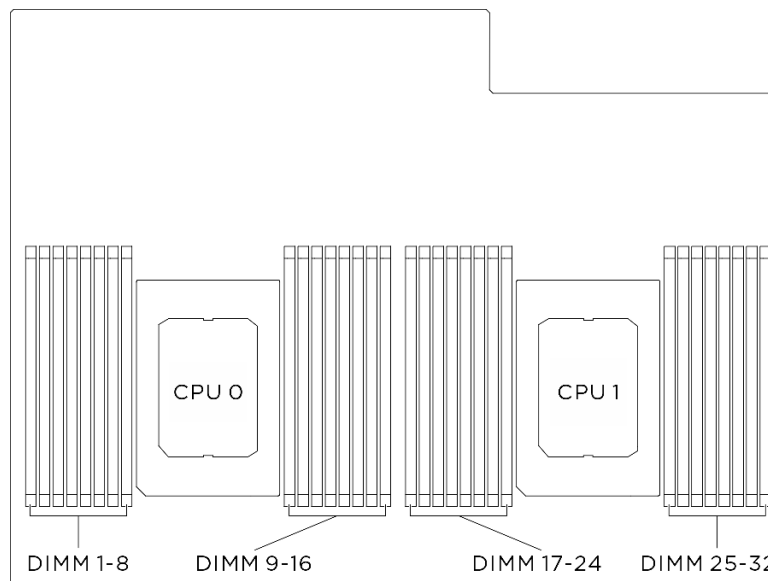
図 60. メモリー・モジュールおよびプロセッサのレイアウト
