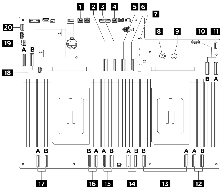
図 191. ケーブル配線用のシステム・ボード・コネクタ
