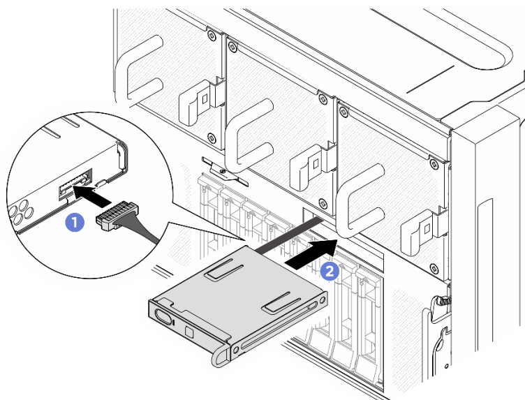
図 51. 内蔵診断パネルの取り付け
