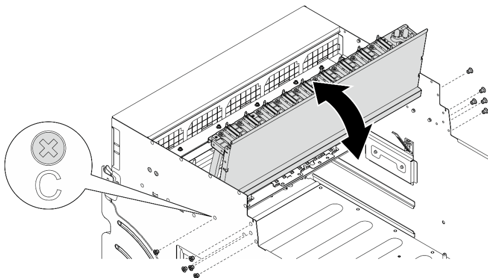
図 117. 前面 PCIe スイッチ・ケーブル・ハーネスをひっくり返す
