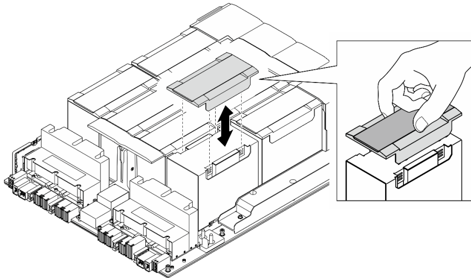
図 145. プラスチック・カバーの取り付け
