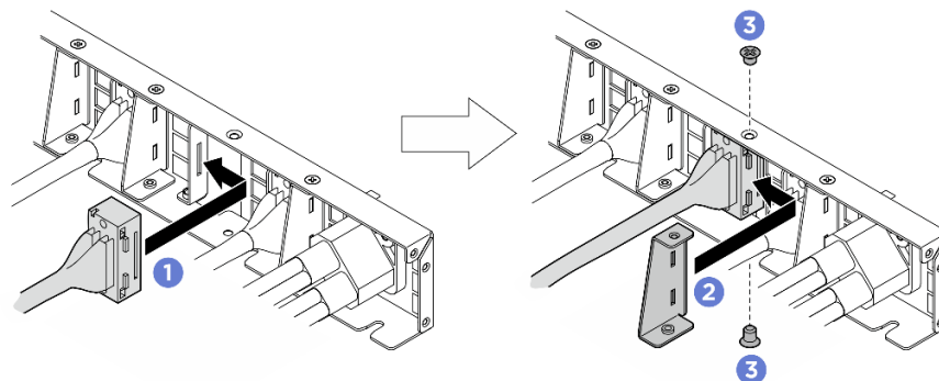
図 175. 前面 I/O モジュール、内蔵診断パネル、GPU 管理、または信号ケーブルの取り付け
