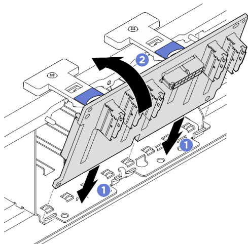
図 112. 2.5 型ドライブ・バックプレーンの取り付け
