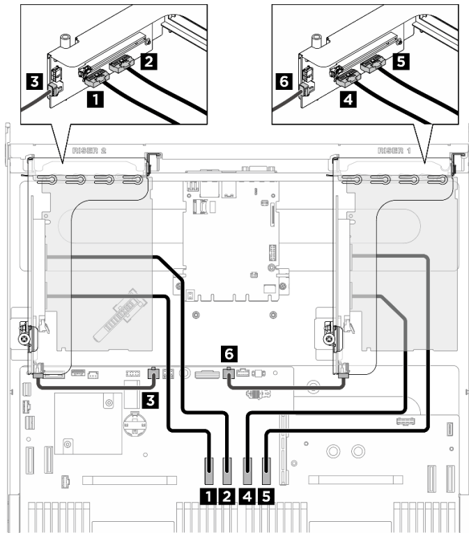
図 192. PCIe ライザーのケーブル配線
