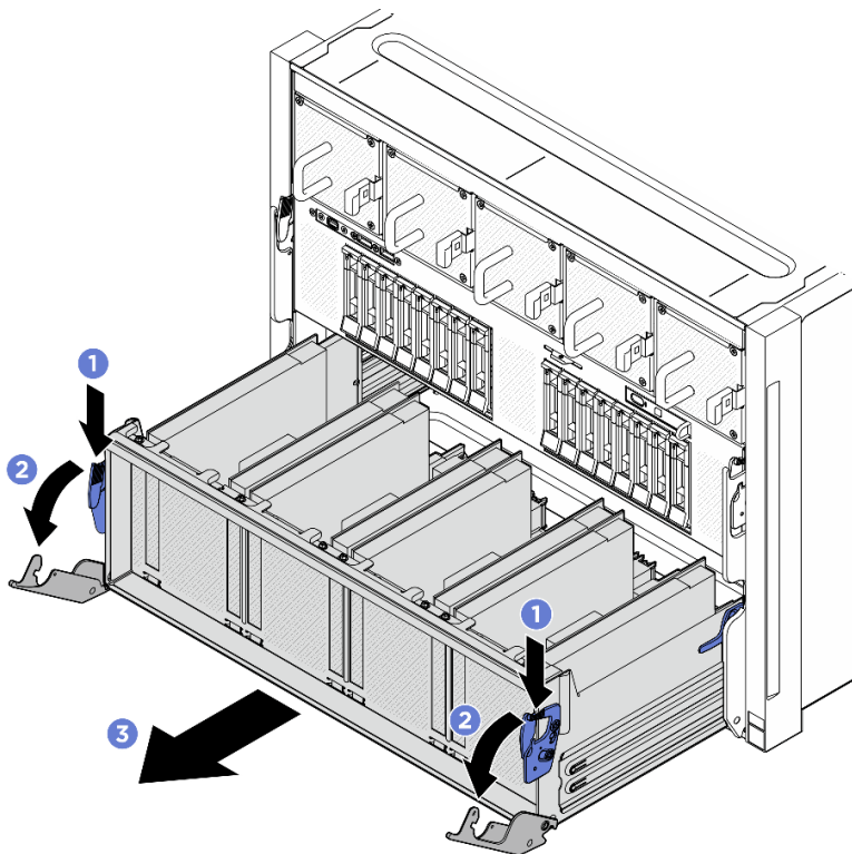
図 134. 停止位置までの PCIe スイッチ・シャトルの取り外し
