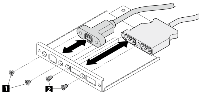
図 162. 前面 I/O モジュール・ケーブルの取り外し
