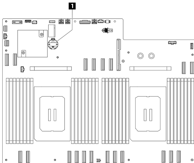
図29. CMOS バッテリーの位置
