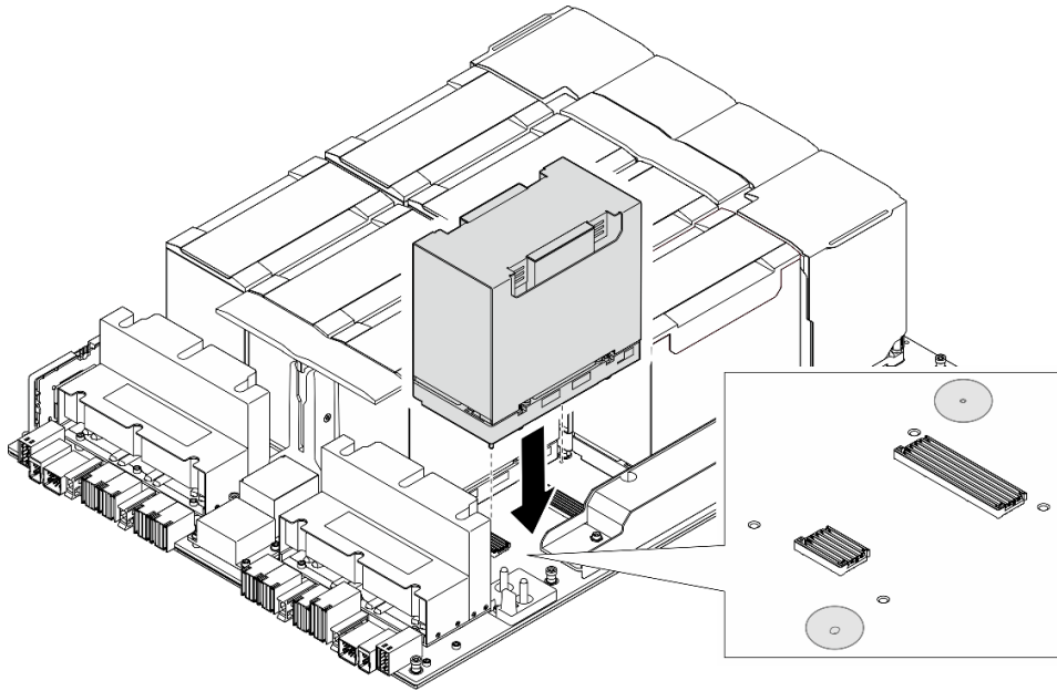
図143. GPU および ヒートシンク・モジュール の取り付け
