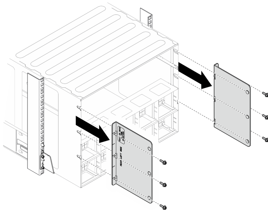
図2. 上部サポート・ブラケットの取り外し
