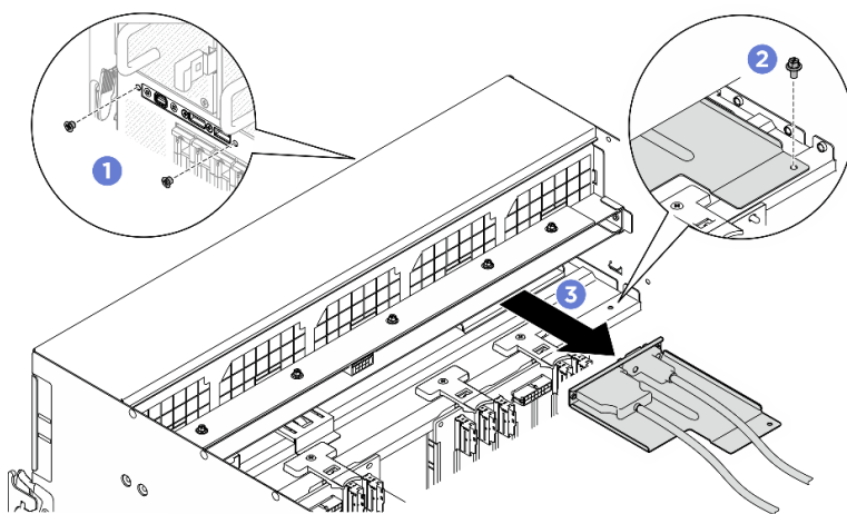
図 161. 前面 I/O モジュールの取り外し
