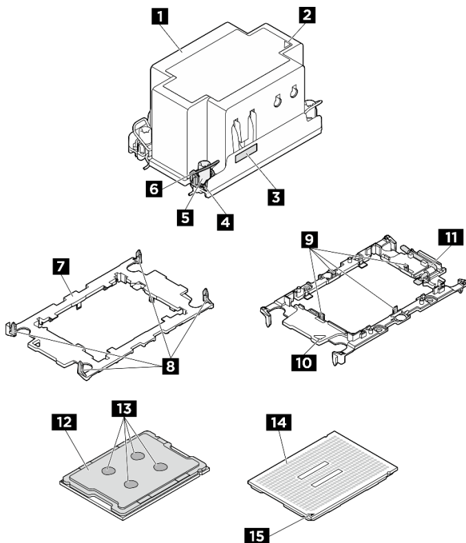
図 86. PHM コンポーネント
