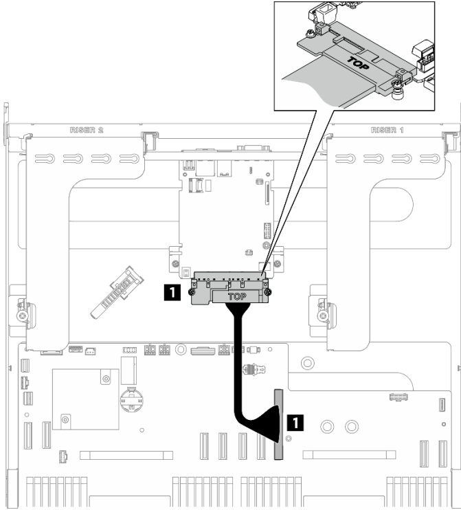
図 199. システム I/O ボードのケーブル配線
