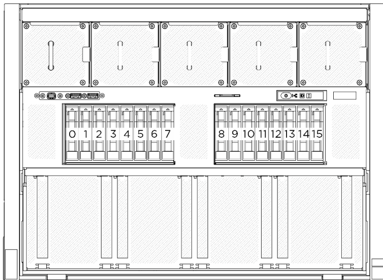
図19. 2.5型ドライブ・ベイ番号
