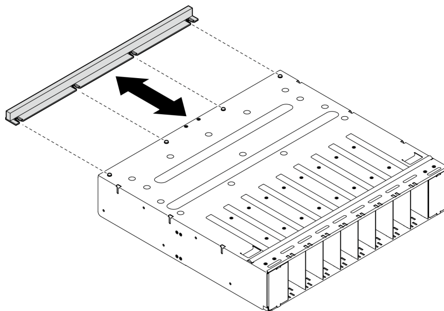
図48. GPU エア・バッフルの取り外し
