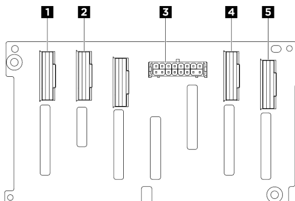
図 182. 2.5 型 NVMe バックプレーン・コネクタ
