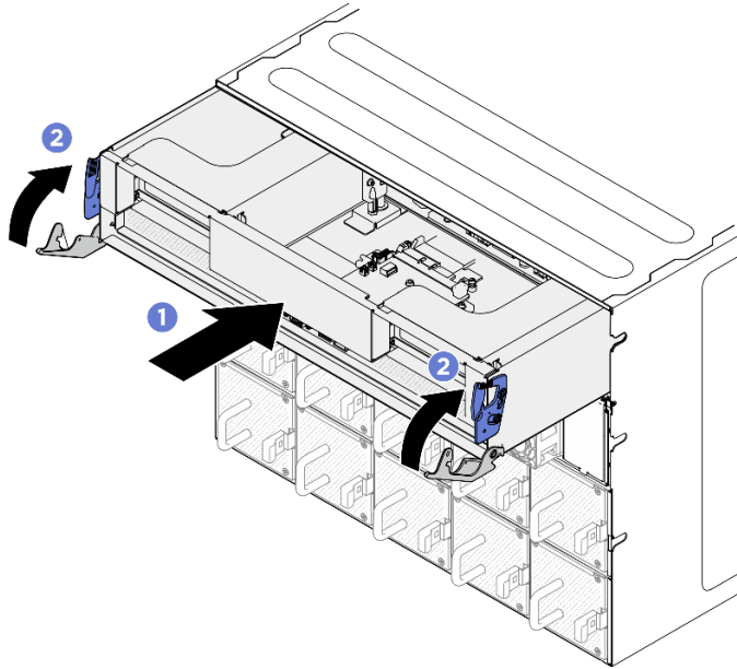
図22. 2U 計算シャトルの取り付け
