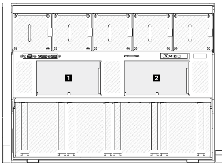
図 109. 2.5 型ドライブ・バックプレーン番号
