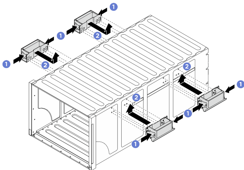
図 10. 4 個のハンドルの取り付け
