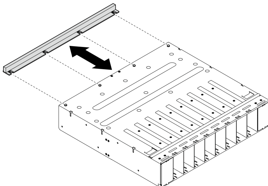
図 49. GPU エアー・バッフルの取り付け
