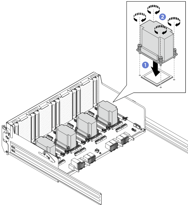
図 154. PCIe スイッチ・ボード・ヒートシンク の取り付け
