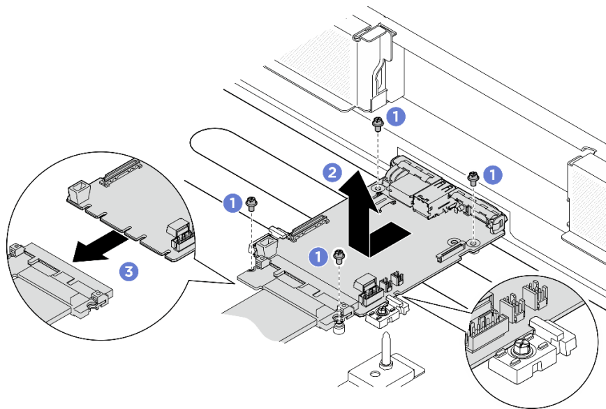
図 83. システム I/O ボードの取り外し
