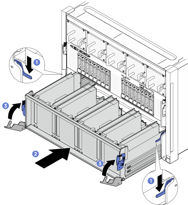
図 124. PCIe スイッチ・シャトルの8U GPU シャトルへの取り付け
