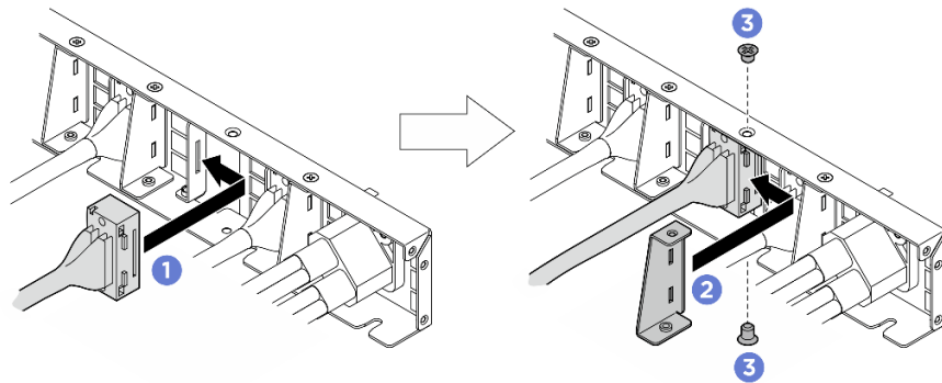
図 173. 前面 I/O モジュール、内蔵診断パネル、GPU 管理、または信号ケーブルの取り外し
