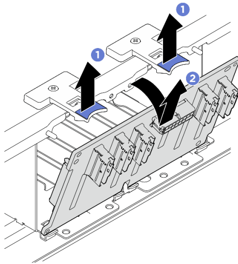
図 110. 2.5 型ドライブ・バックプレーンの取り外し
