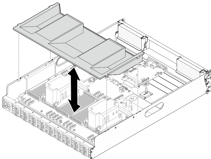
図 82. プロセッサ・エアー・バッフルの取り付け
