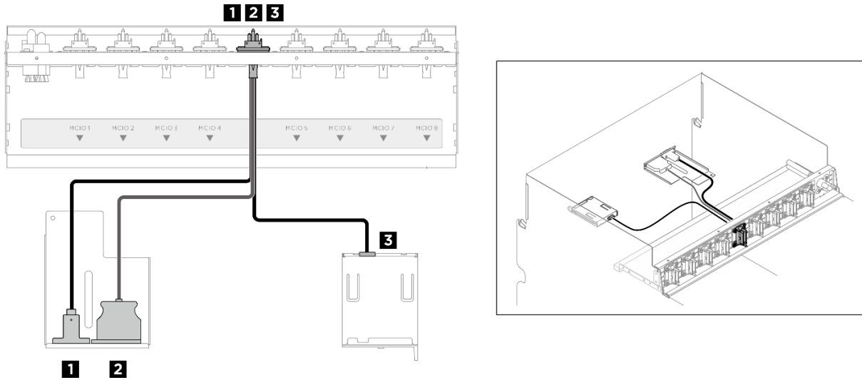
図 198. 前面 I/O モジュールおよび内蔵診断パネルのケーブル配線
