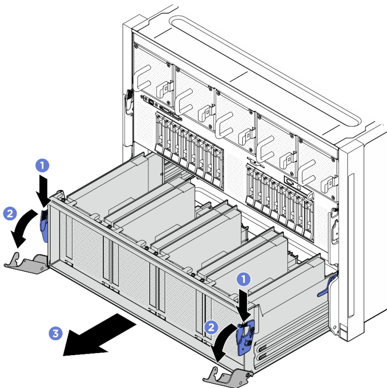
図 125. 停止位置までの PCIe スイッチ・シャトルの取り外し
