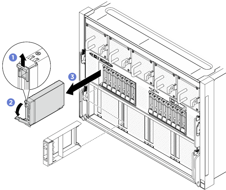
図 18. 2.5 型ホット・スワップ・ドライブの取り外し
