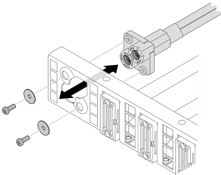
図 174. 電源ケーブルの取り外し
