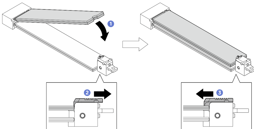
図 57. 上段の M.2 ドライブの取り付け
