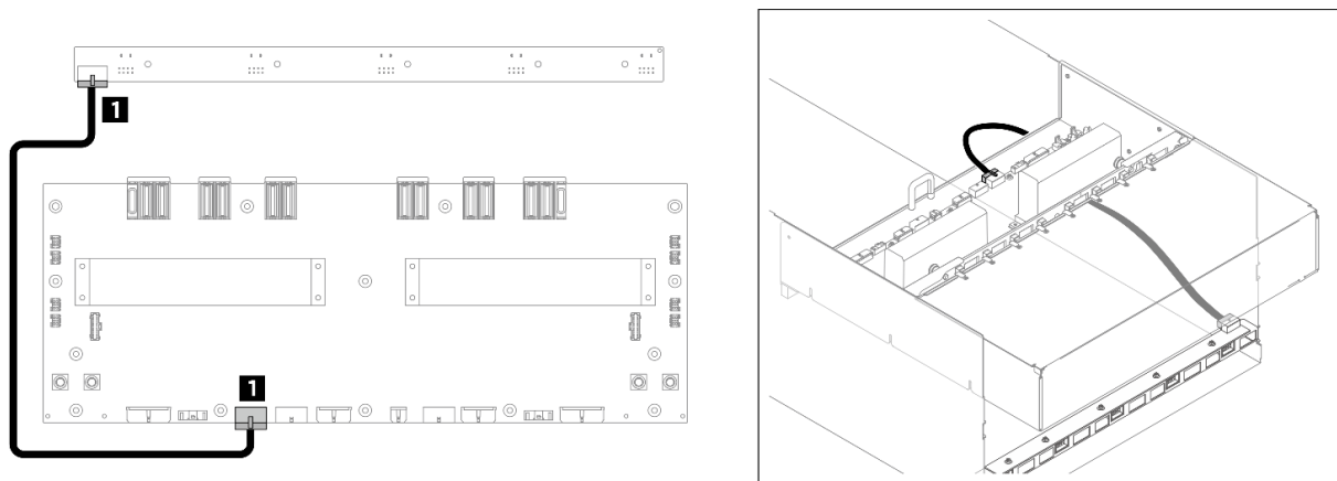
図 196. 背面ファン制御ボード (下部) ケーブル配線
