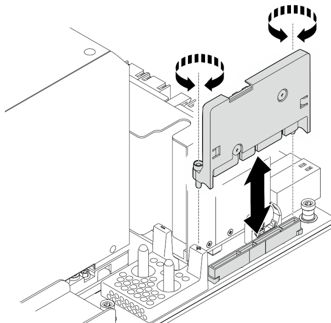
図 146. HMC カードの取り外し
