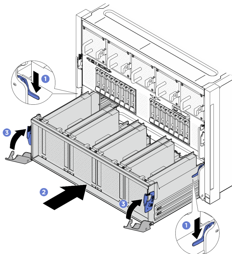
図 139. PCIe スイッチ・シャトルの 8U GPU シャトルへの取り付け
