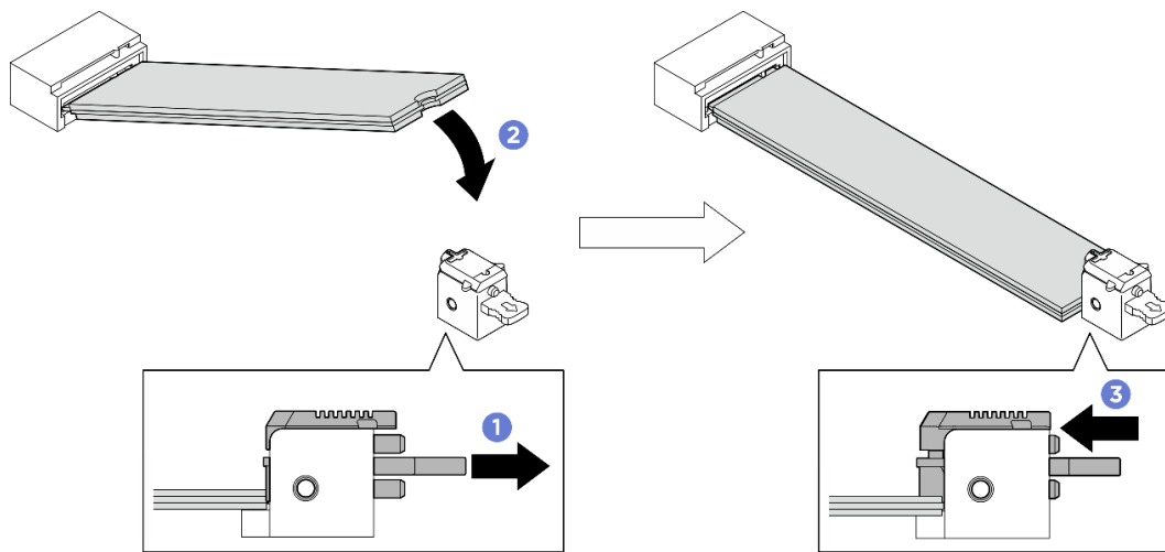
図 56. 下段の M.2 ドライブの取り付け
