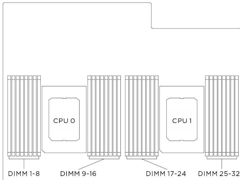
図58. メモリー・モジュールおよびプロセッサのレイアウト
