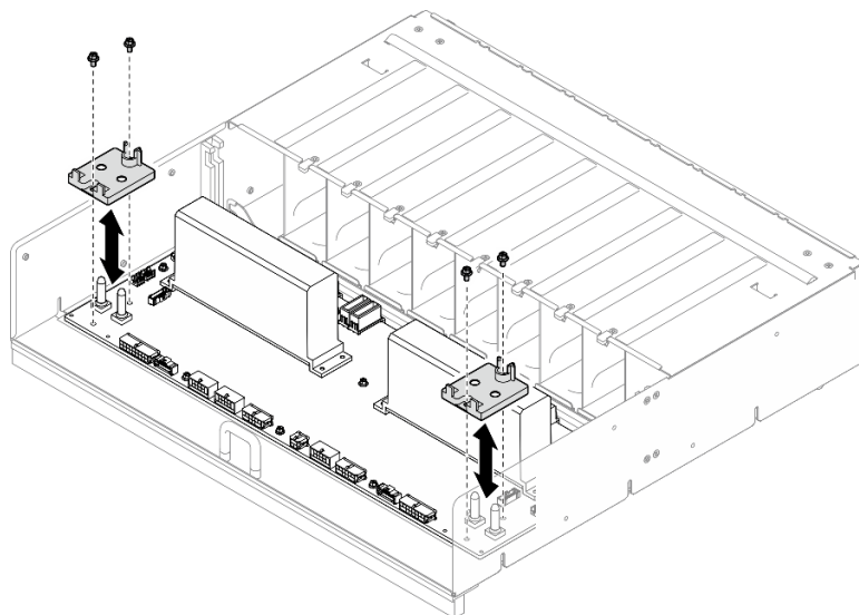
図 73. ケーブル保持具の取り外し
