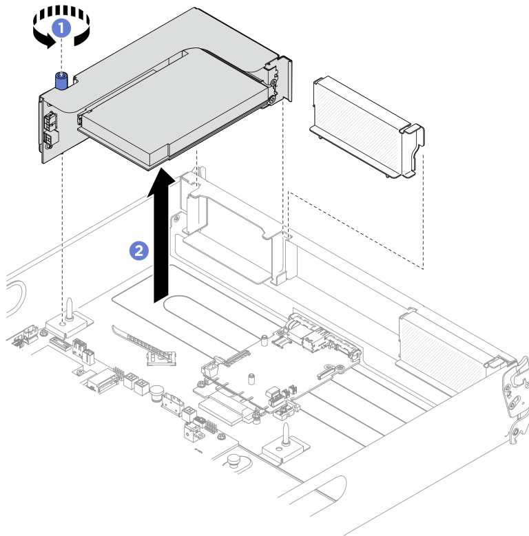
図 65. PCIe ライザー・アセンブリーの取り外し
