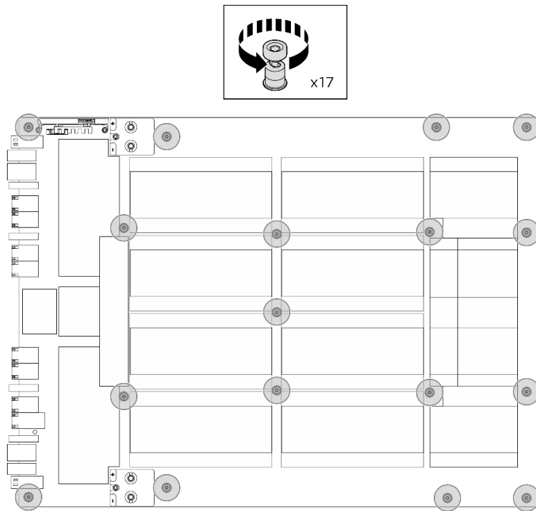
図 127. ねじの取り外し
