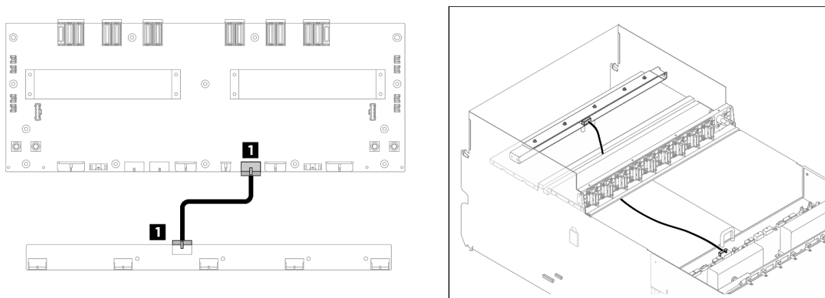
図 194. 前面ファン制御ボードのケーブル配線
