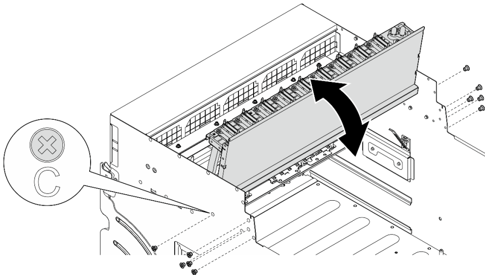
図 138. 前面 PCIe スイッチ・ケーブル・ハーネスをひっくり返す
