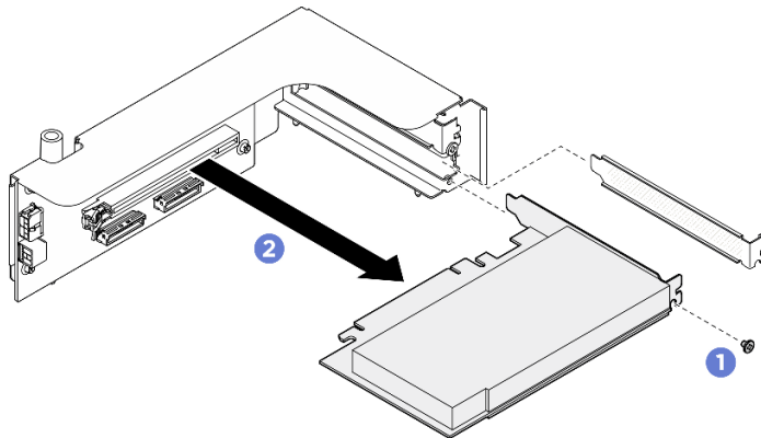
図 159. 背面 PCIe アダプターの取り外し
