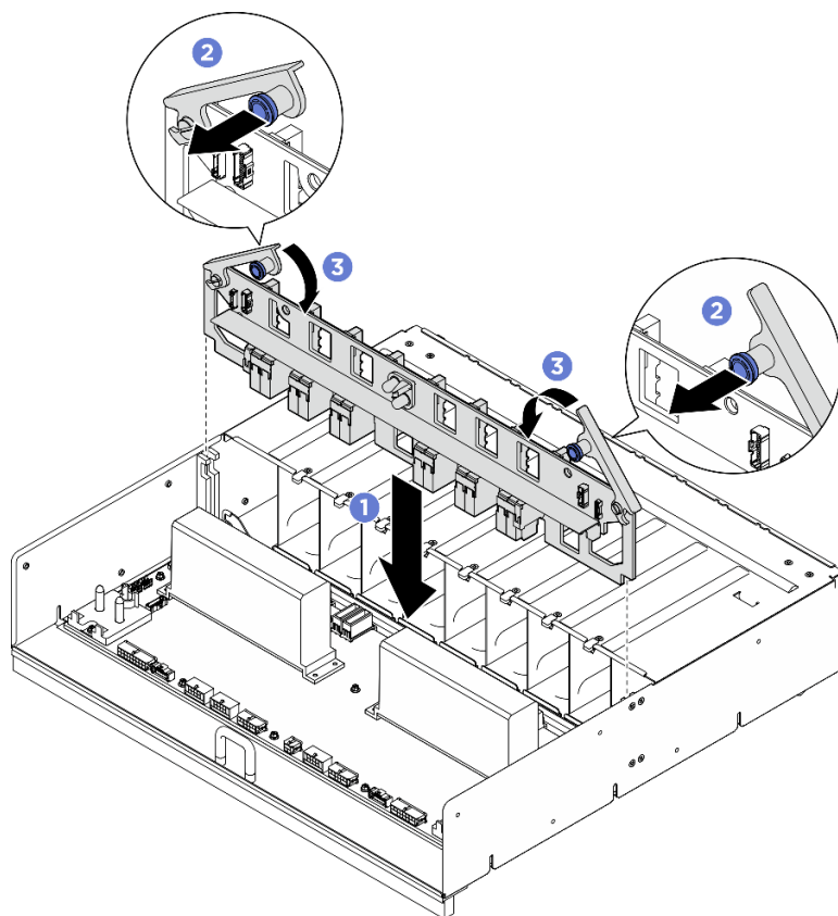
図 100. PSU 変換コネクターの取り付け
