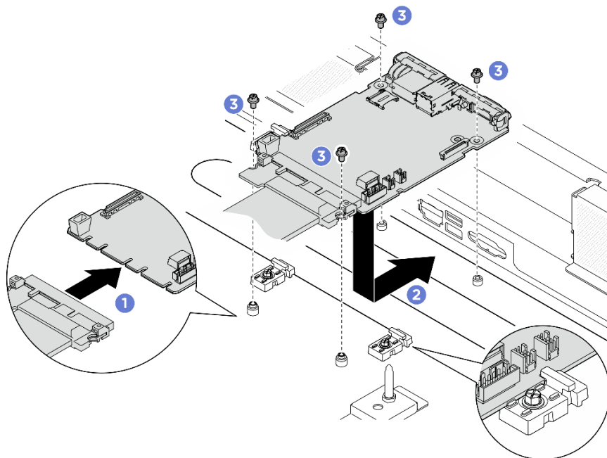
図84. システム I/O ボードの取り付け
