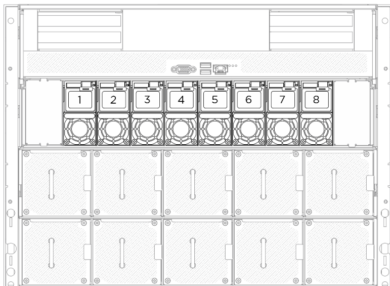
図79. パワー・サプライのベイ番号付け
