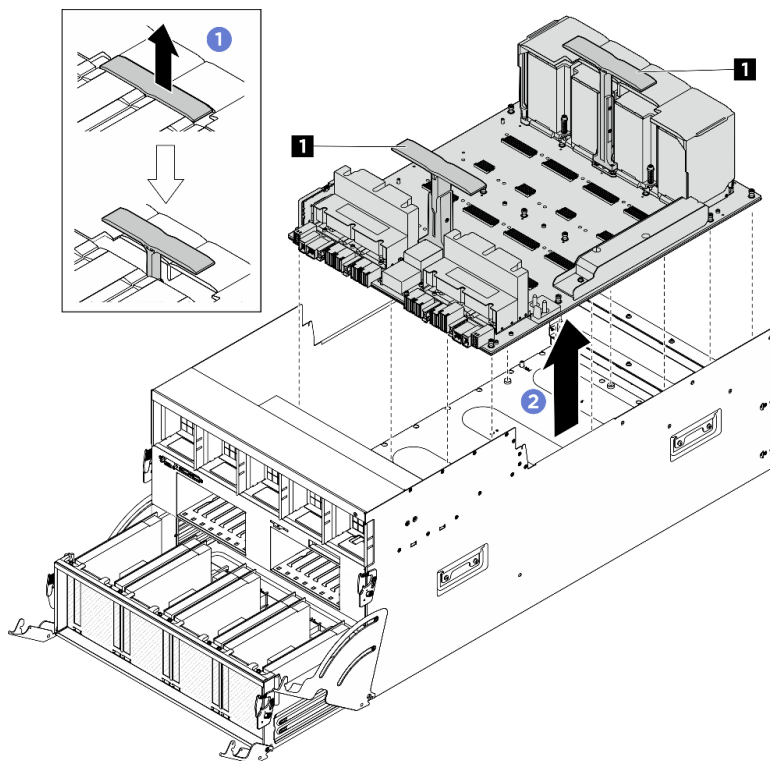
図 119. GPU ベースボードの取り外し
