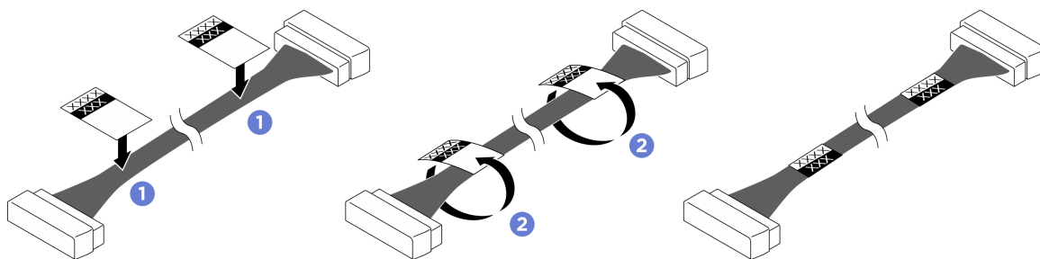
図46. ラベルの貼り付け
