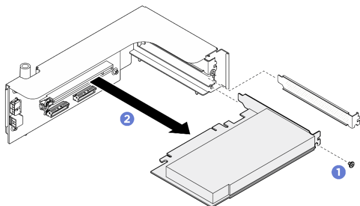
図 66. 背面 PCIe アダプターの取り外し
