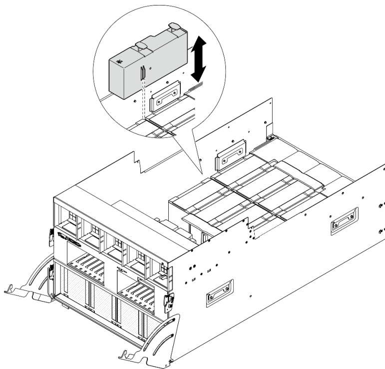
図 114. GPU エアー・ダクトの取り外し
