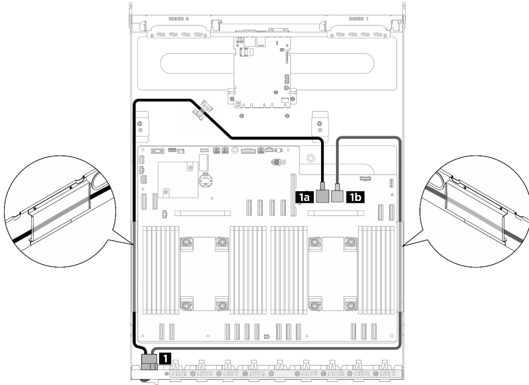
図 200. 電源ケーブルの電源ケーブル配線
