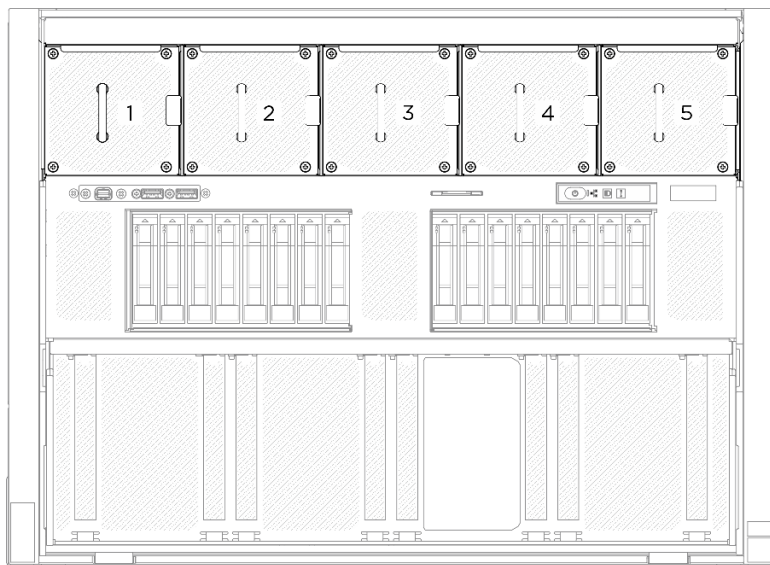
図 31. 前面ファン番号
