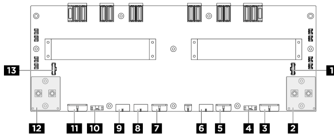
図 189. 分電盤コネクタ
