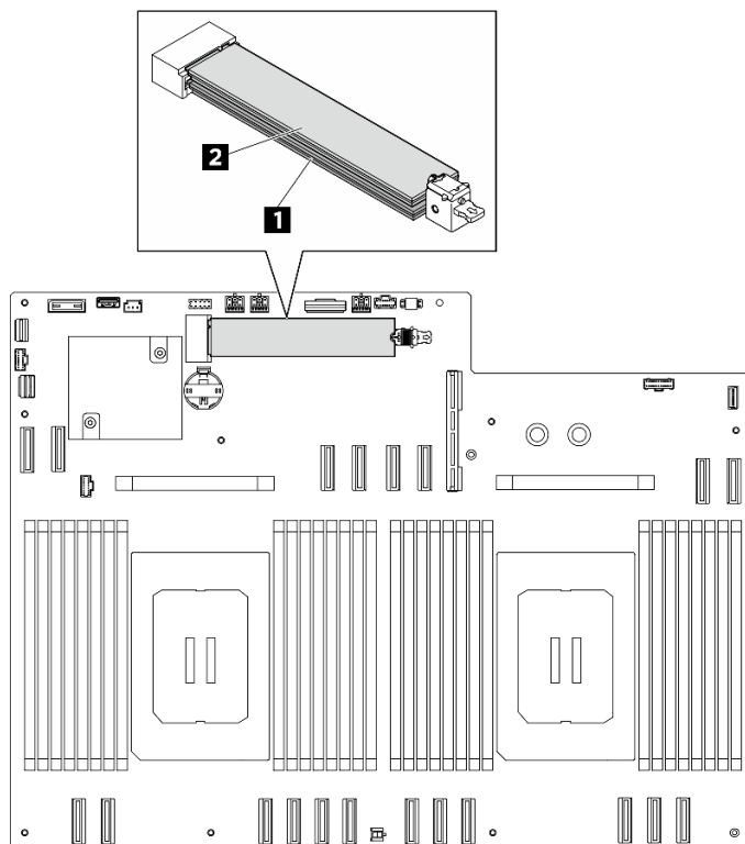
図 52. M.2 ドライブ・スロット
