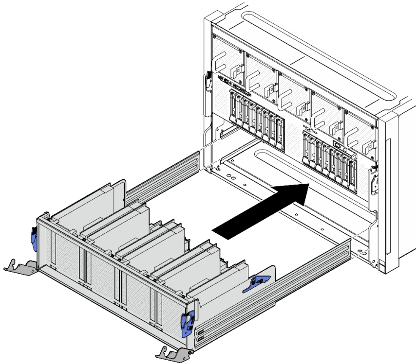
図 180. 停止位置への PCIe スイッチ・シャトルの取り付け
