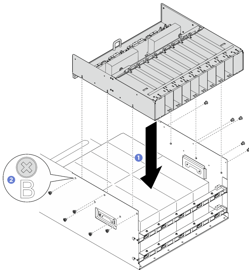
図 72. 電源複合システムの取り付け
