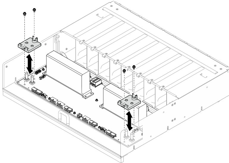
図 99. ケーブル保持具の取り付け
