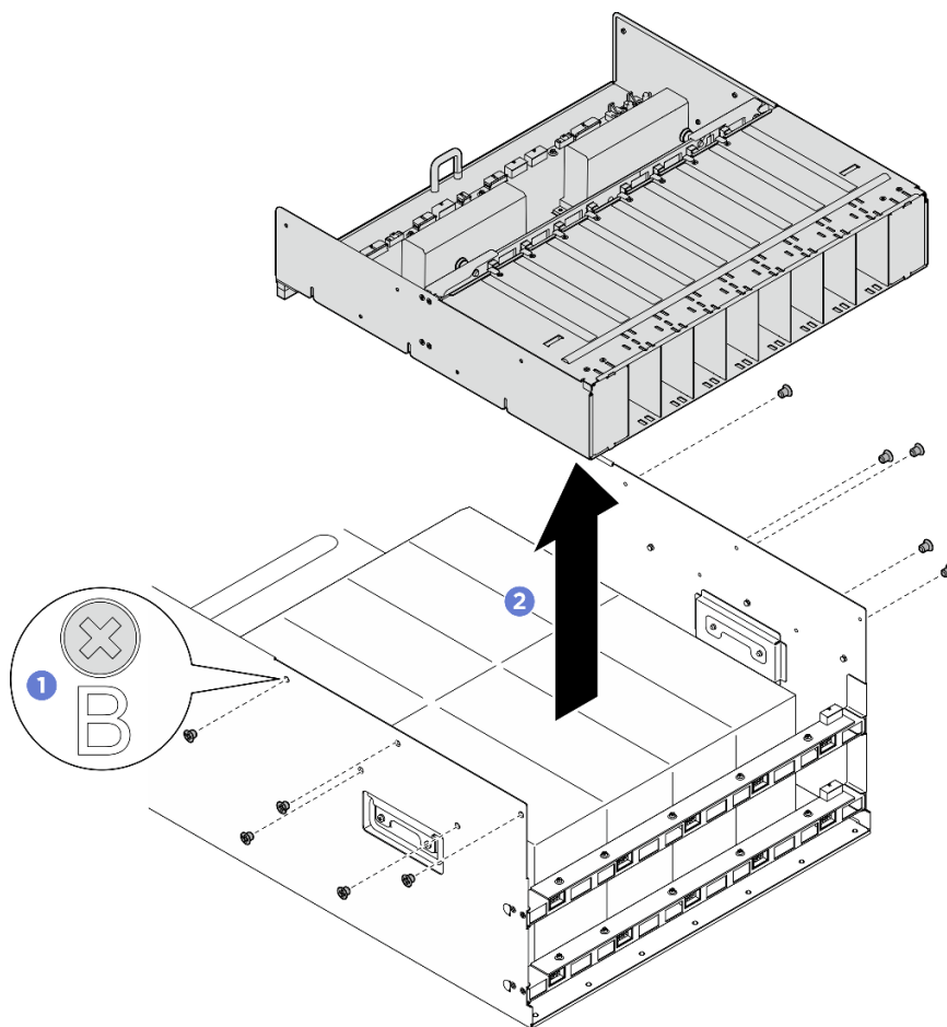
図 71. 電源複合システムの取り外し
