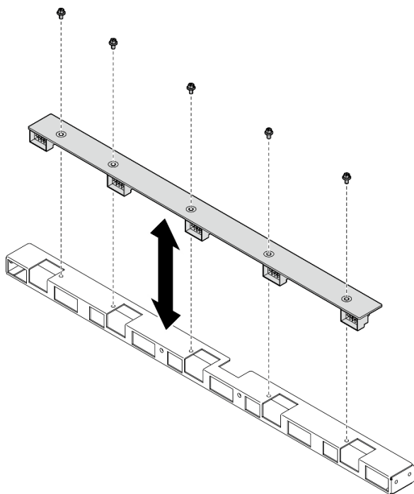
図43. 背面ファン制御ボードの取り外し
