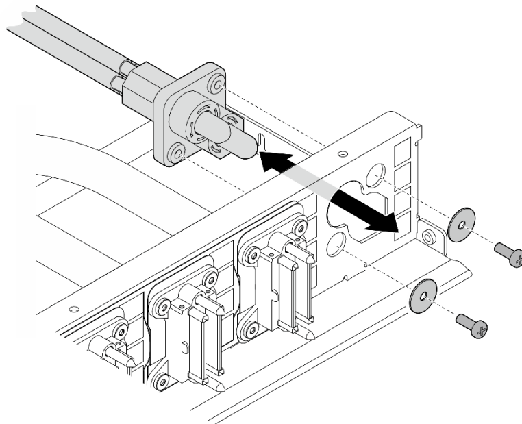
図 168. 電源ケーブルの取り付け
