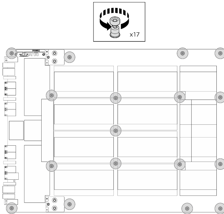
図118. ねじの取り外し
