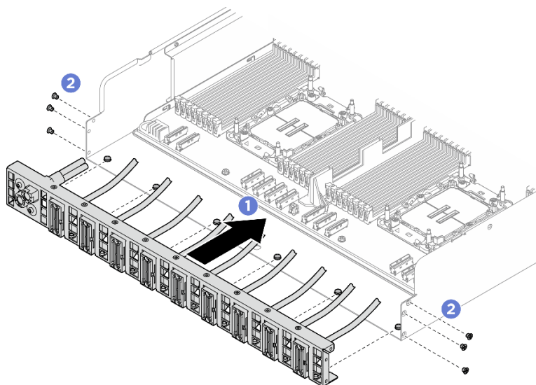
図 177. 背面 PCIe スイッチ・ケーブル・ハーネス の取り付け
