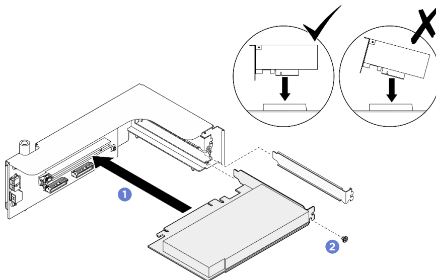
図 160. 背面 PCIe アダプターの取り付け
