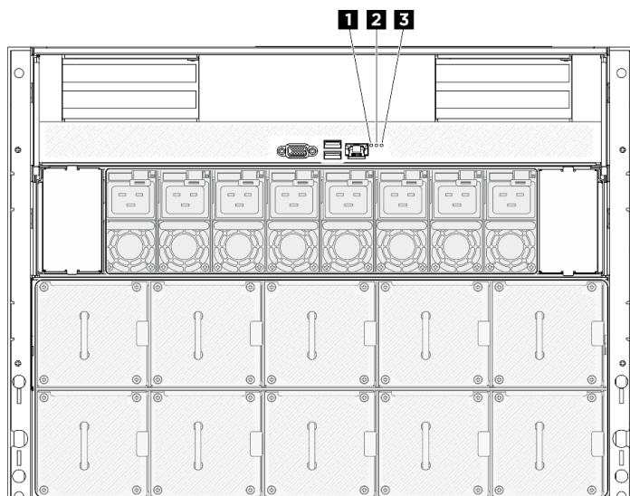
図 214. 背面図のシステム LED
