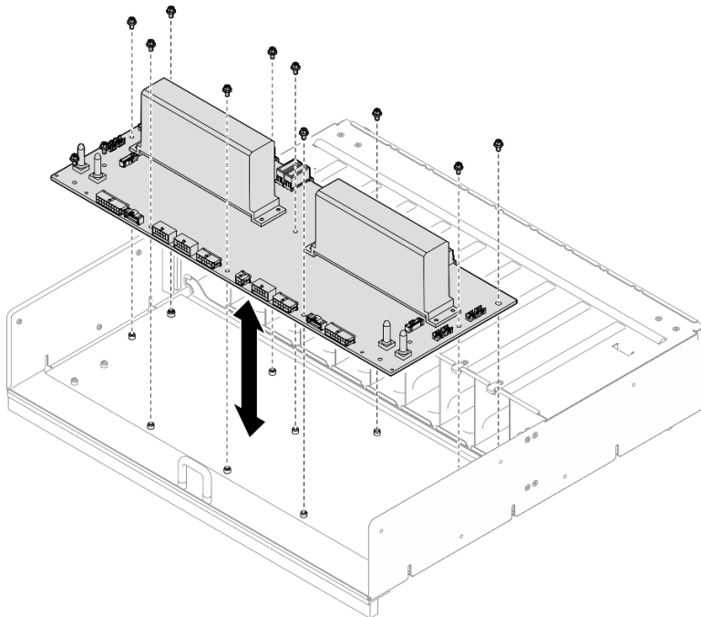
図97. 分電盤の取り外し
