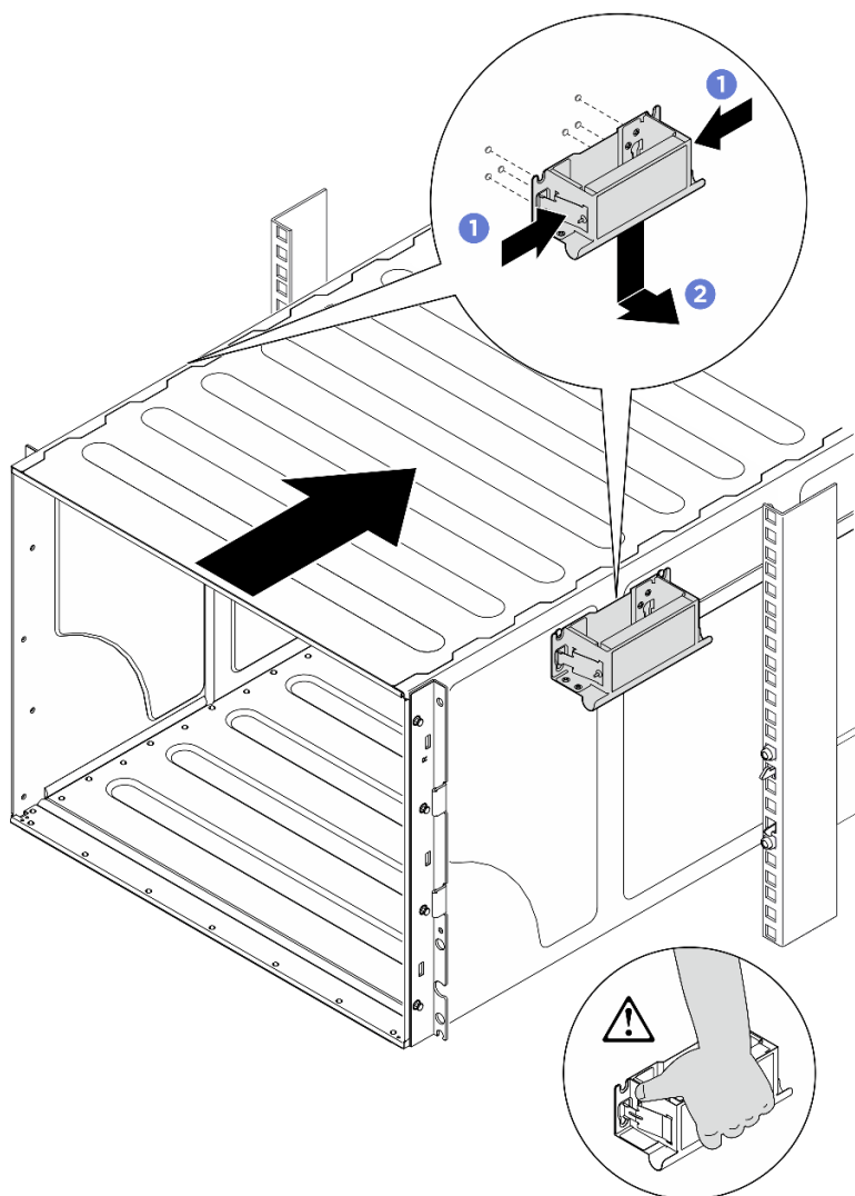
図12. 前面ハンドルの取り外し
