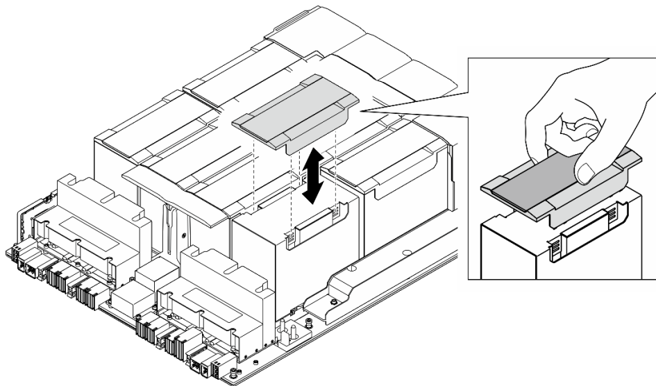
図 142. プラスチック・カバーの取り外し
