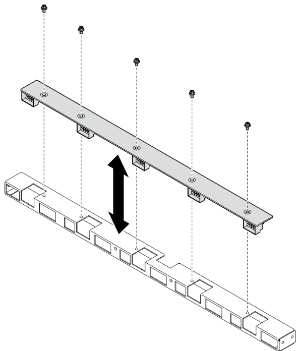
図 39. 前面ファン制御ボードの取り付け
