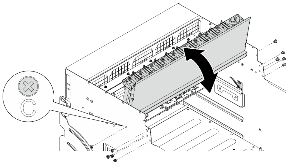
図 135. 前面 PCIe スイッチ・ケーブル・ハーネスをひっくり返す
