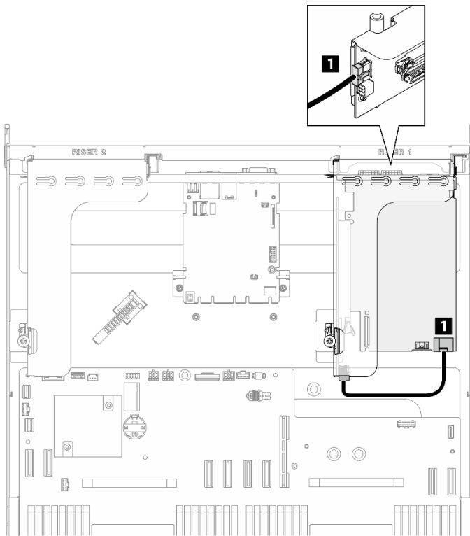
図 193. DPU 電源ケーブル配線
