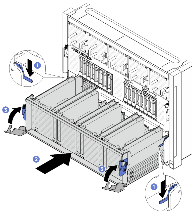
図 158. PCIe スイッチ・シャトルの 8U GPU シャトルへの取り付け
