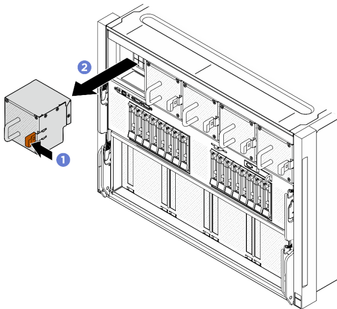
図33. ホット・スワップ・ファンの取り外し
