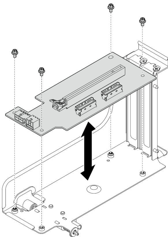
図 67. PCIe ライザー・カードの取り外し
