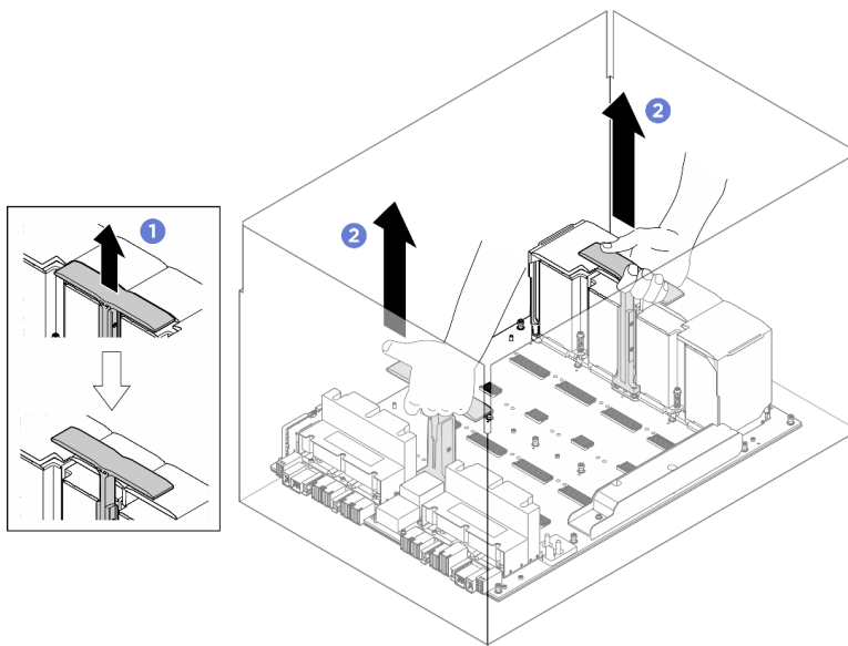
図 120. パッケージ・ボックスからの GPU ベースボードの取り外し
