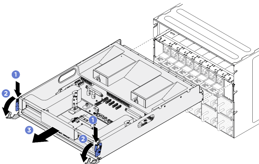
図 21. 2U 計算シャトルの取り外し
