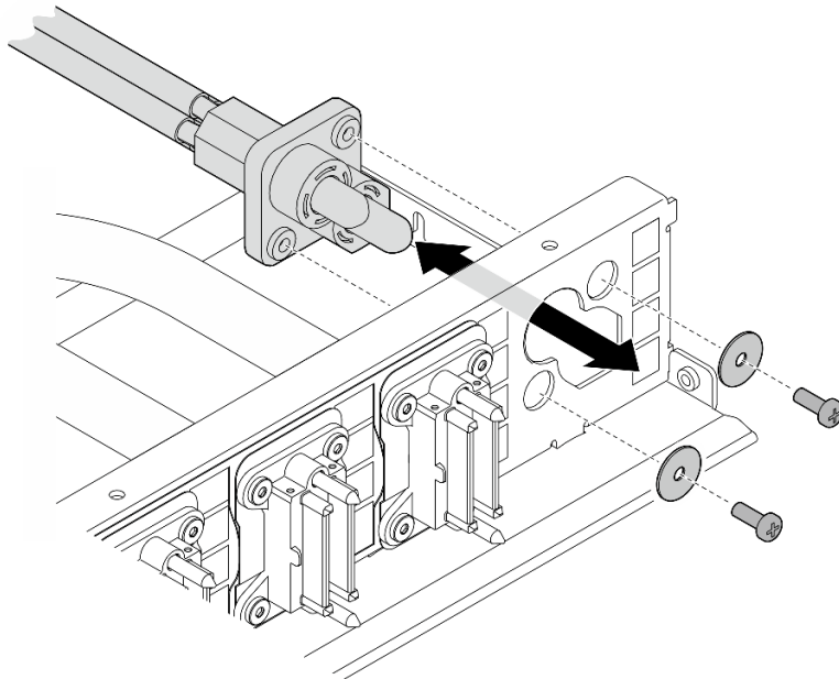
図 165. 電源ケーブルの取り外し
