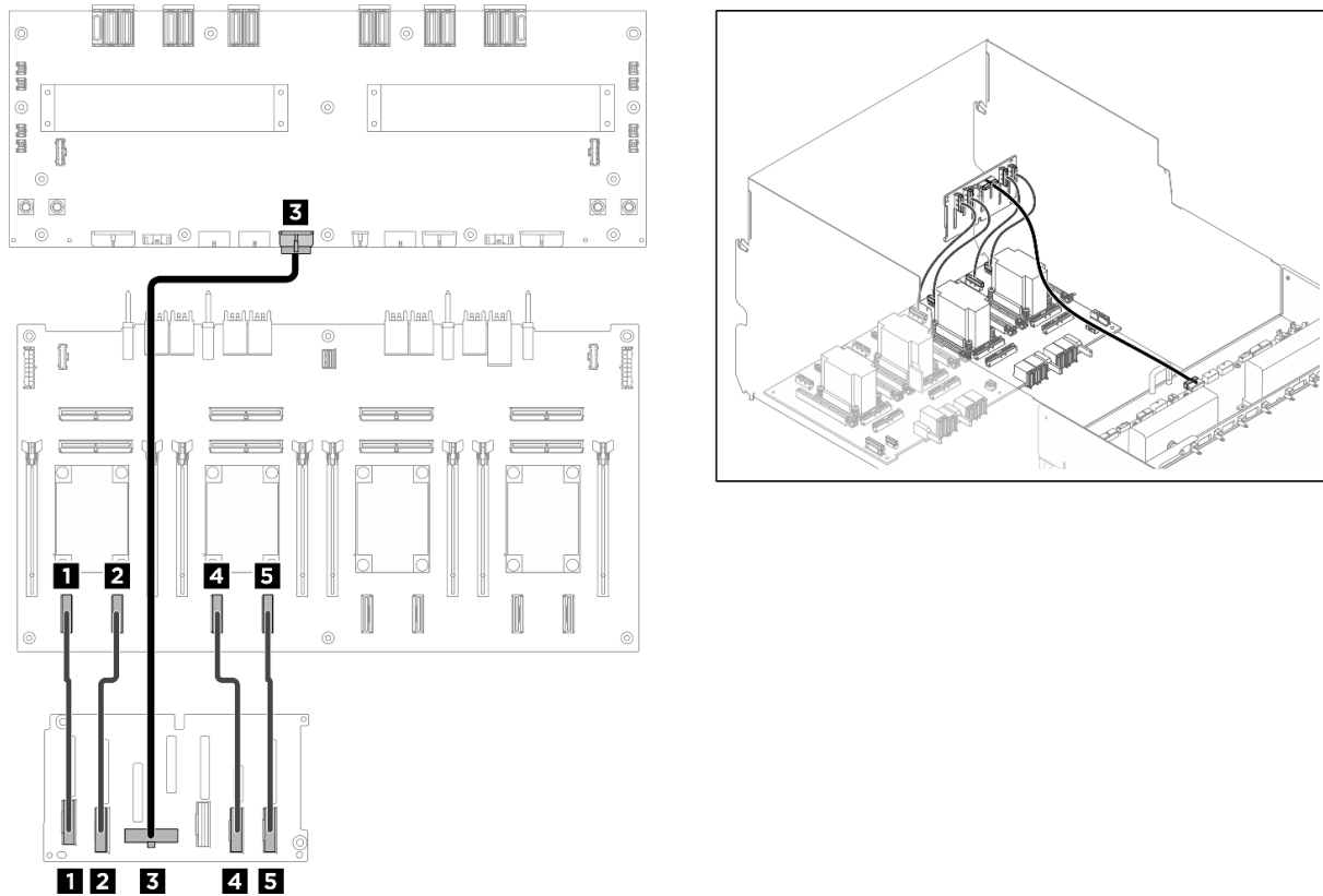
図 202. バックプレーン 1 のケーブル配線
