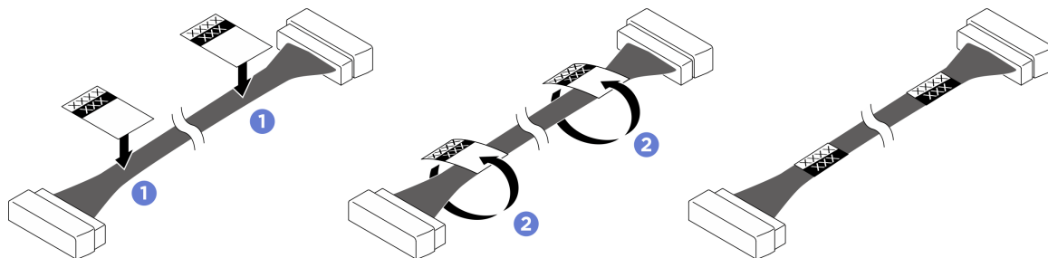
図 69. ラベルの貼り付け
