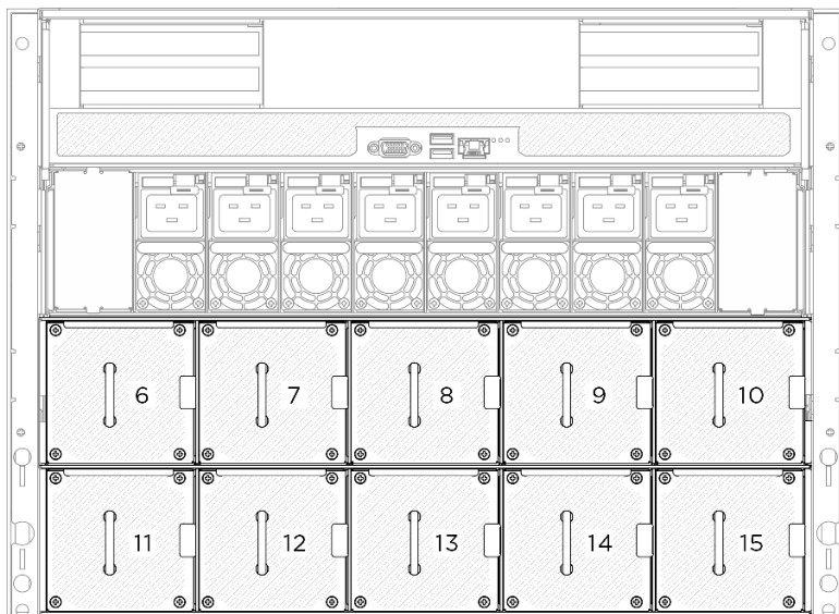
図 32. 背面ファン番号
