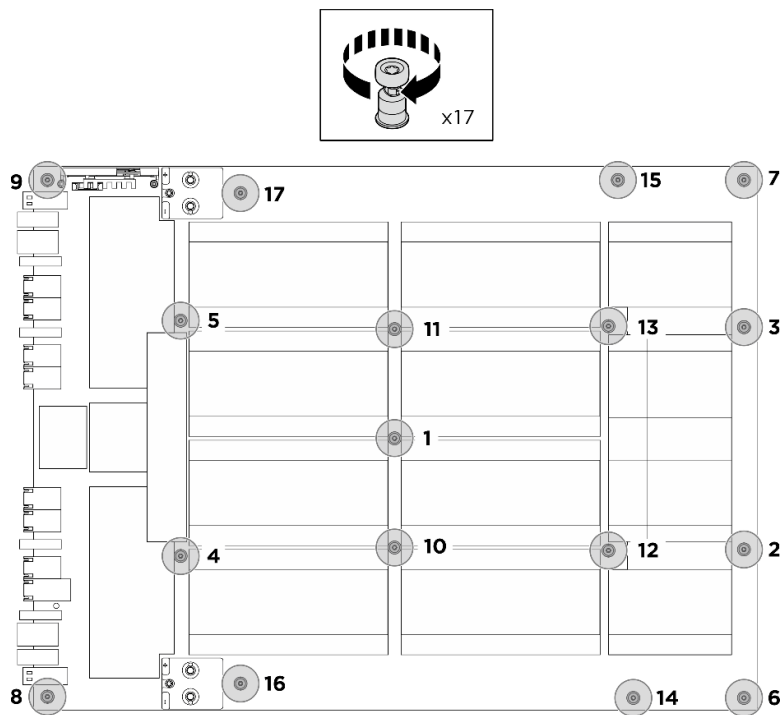
図 131. ねじの取り付け
