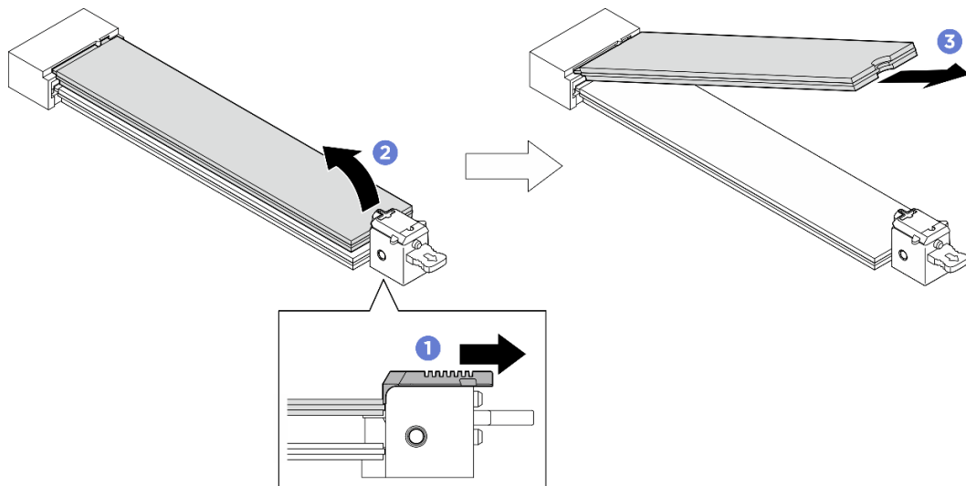
図 53. 上段の M.2 ドライブの取り外し
