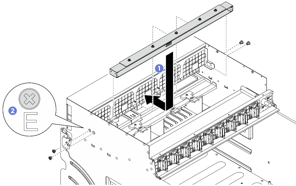
図40. 前面ファン制御ボード・アセンブリーの取り付け
