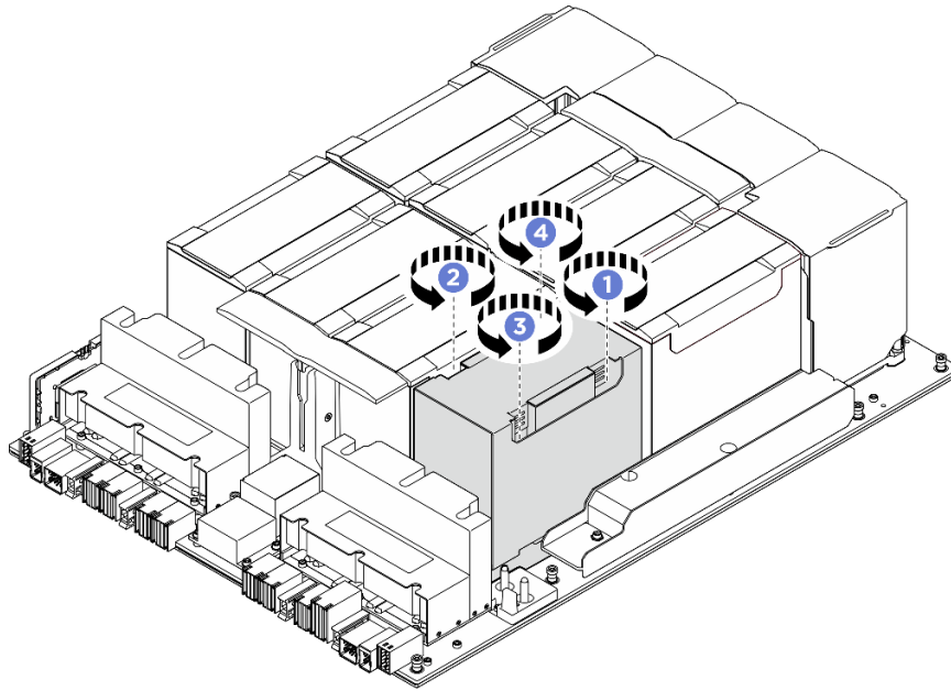
図 144. ねじの締め付け順序
