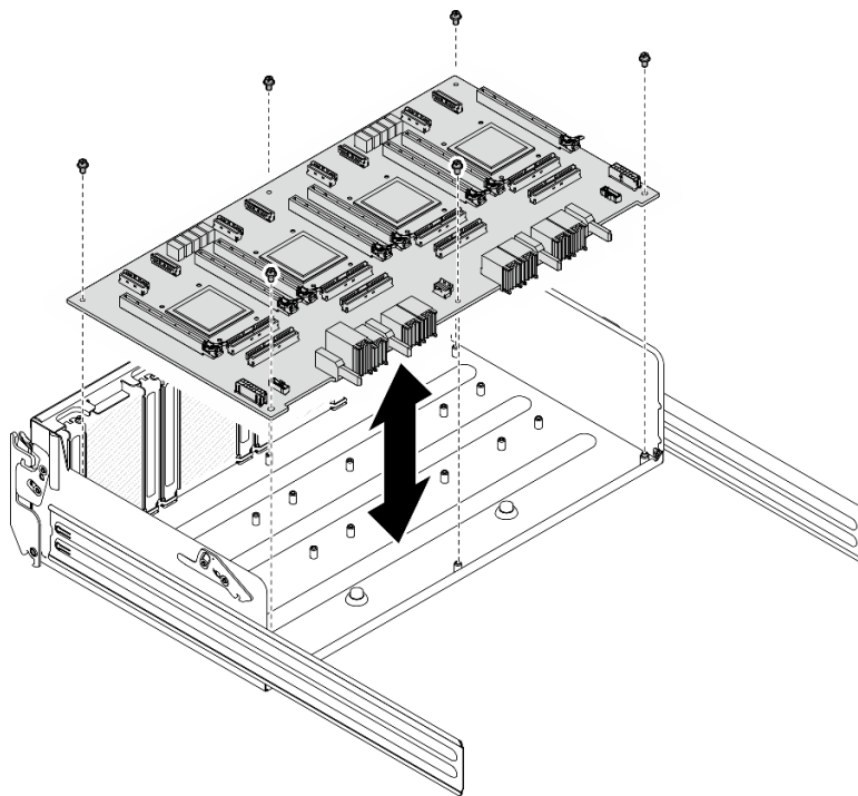
図 151. PCIe スイッチ・ボードの取り外し
