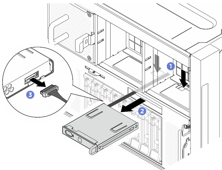
図 50. 内蔵診断パネルの取り外し
