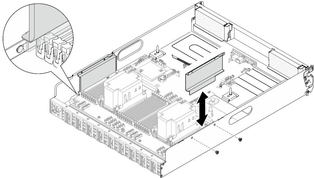
図108. ケーブル・ガイドの取り付け
