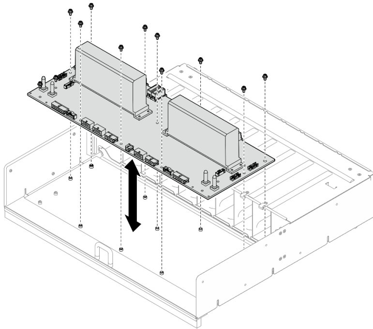
図 75. 分電盤の取り付け
