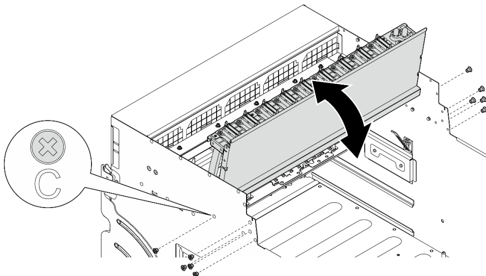
図 123. 前面 PCIe スイッチ・ケーブル・ハーネスをひっくり返す
