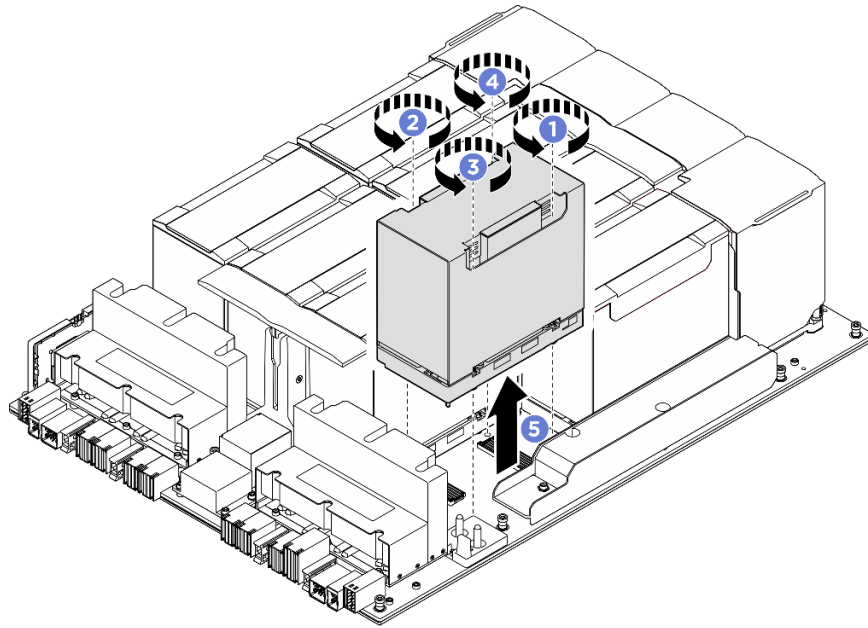
図 141. GPU および ヒートシンク・モジュールの取り外し
