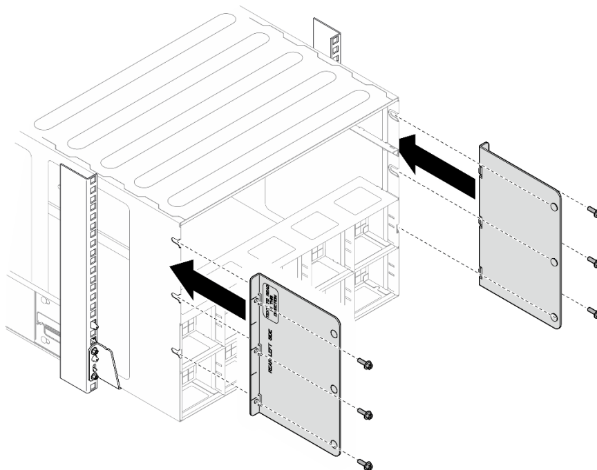
図 16. 上部サポート・ブラケットの取り付け
