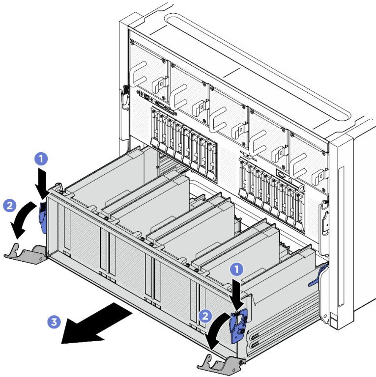
図 178. 停止位置までの PCIe スイッチ・シャトルの取り外し
