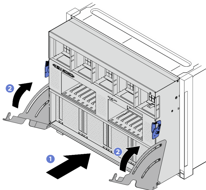
図 24. 8U GPU シャトルの取り付け
