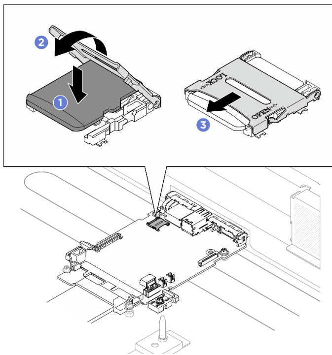
図 63. MicroSD カードの取り付け
