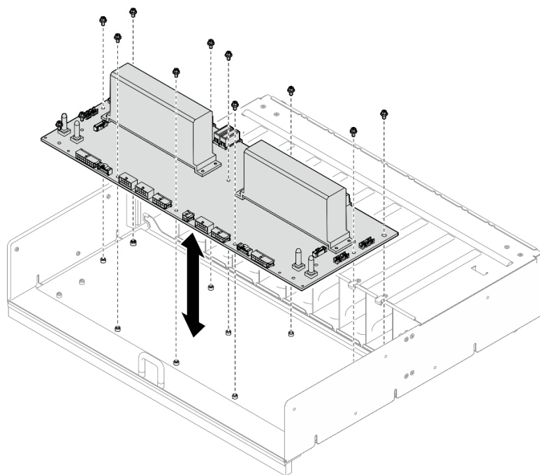
図 98. 分電盤の取り付け
