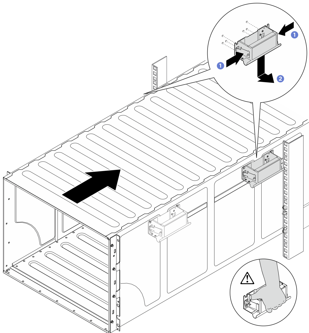
図11. 後部ハンドルの取り外し
