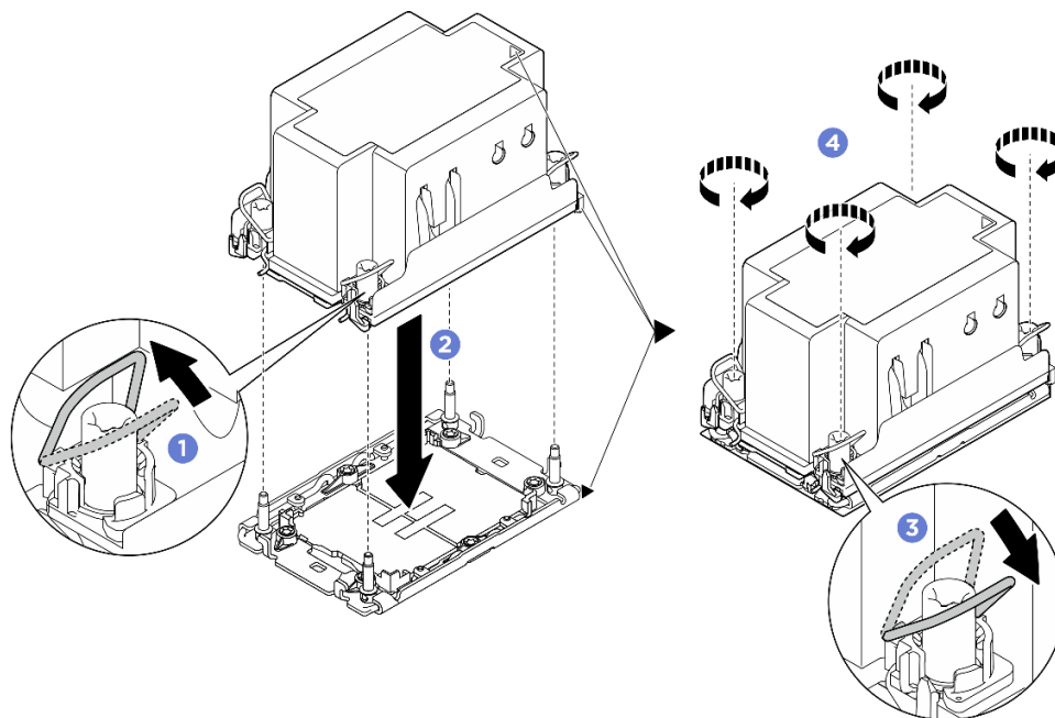
図94. PHM の取り付け
