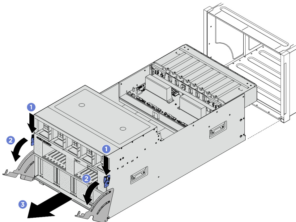
図23. 8U GPU シャトルの取り外し
