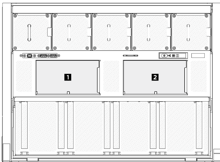
図 111. 2.5 型ドライブ・バックプレーン番号
