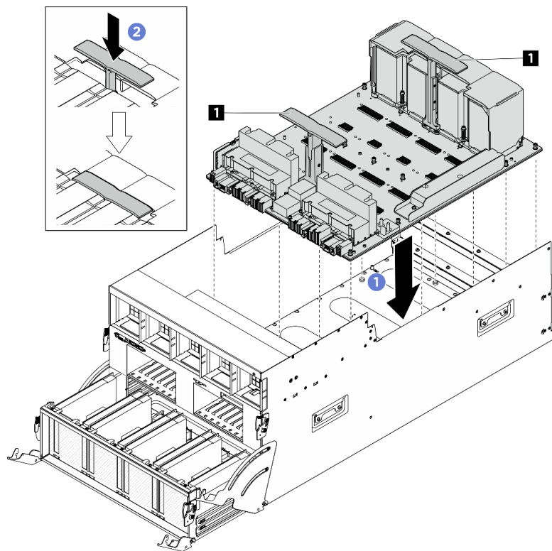
図 121. GPU ベースボード の取り付け
