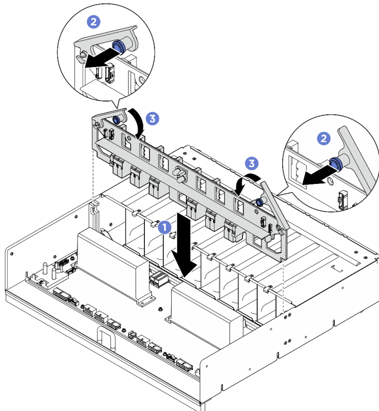
図 102. PSU 変換コネクタの取り付け
