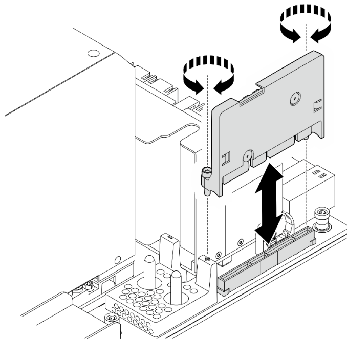
図 147. HMC カードの取り付け
