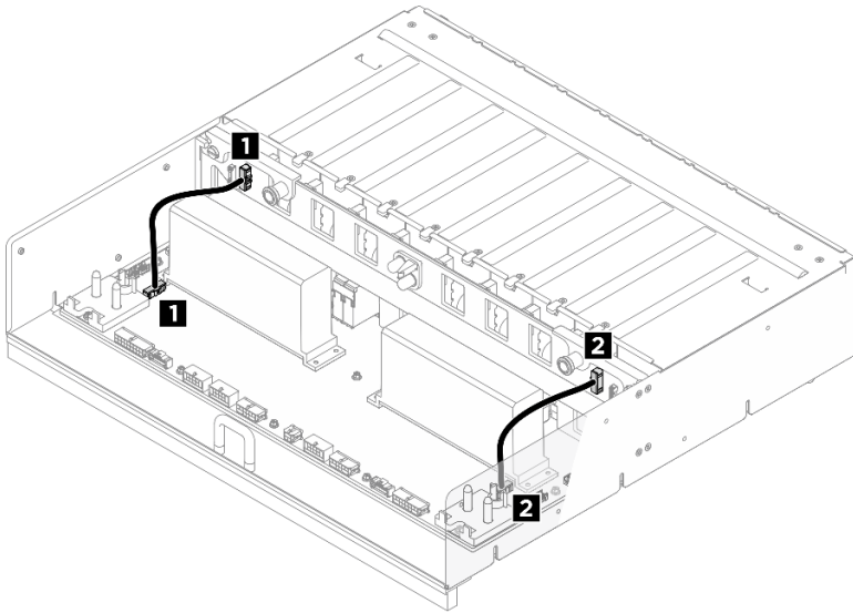
図 201. PSU 変換コネクタのケーブル配線
