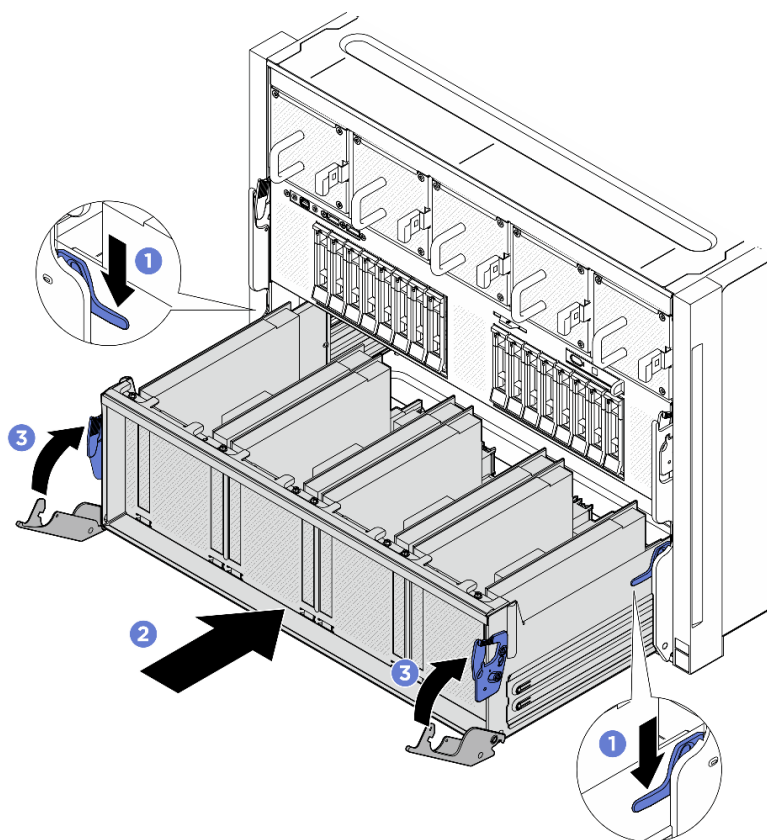
図 133. PCIe スイッチ・シャトルの8U GPU シャトルへの取り付け
