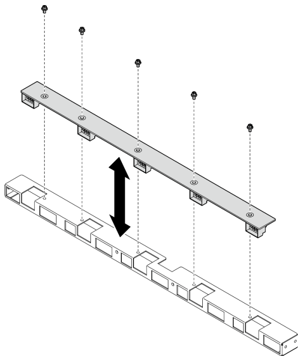
図 44. 背面ファン制御ボードの取り付け
