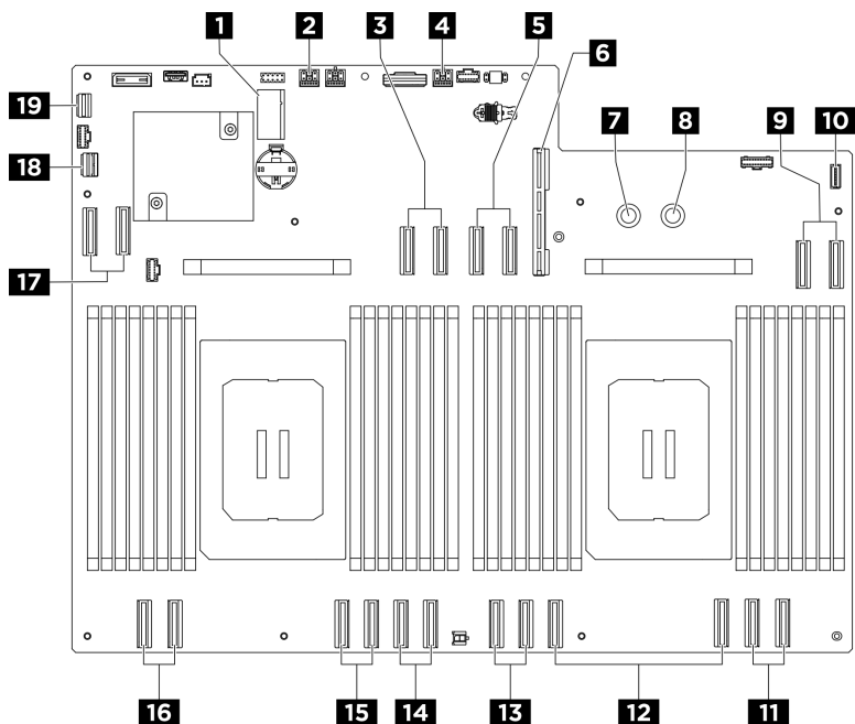
図 211. システム・ボード・コネクタ
