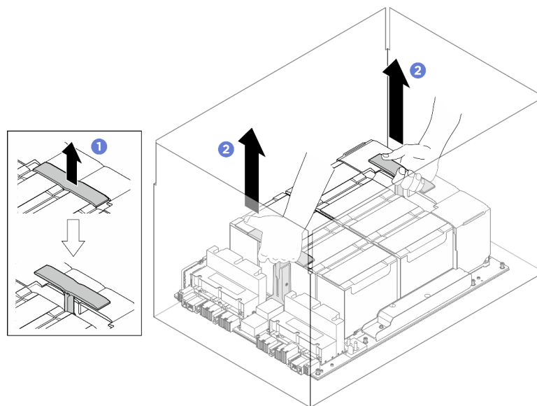
図 129. パッケージ・ボックスからの GPU 複合システムを取り外し
