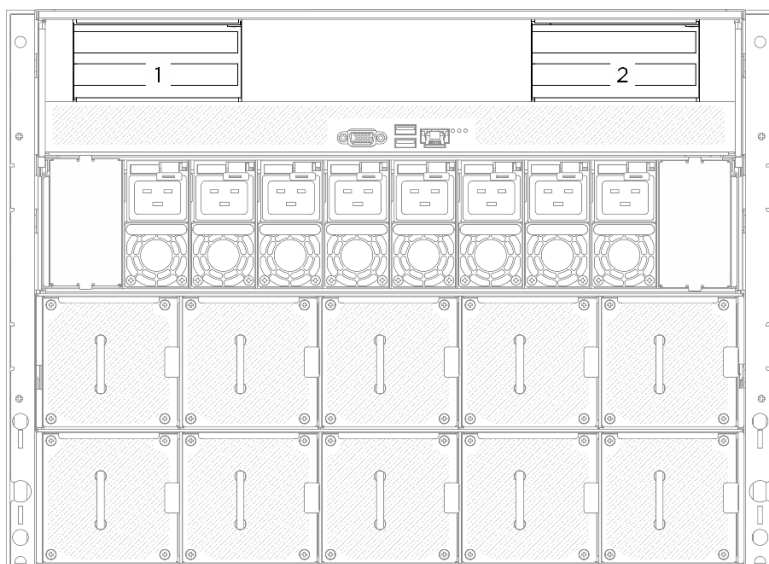
図 64. PCIe ライザーの位置
