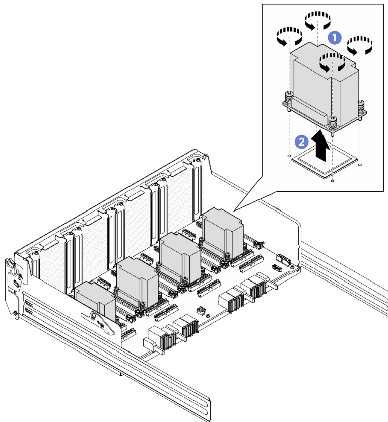
図 150. PCIe スイッチ・ボード・ヒートシンクの取り外し
