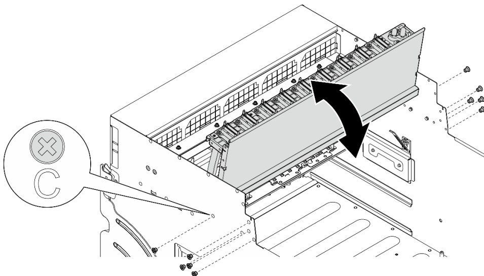
図 126. 前面 PCIe スイッチ・ケーブル・ハーネスをひっくり返す
