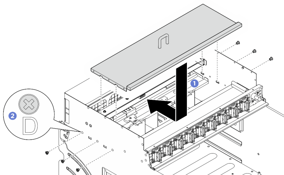
図 149. I/O カバーの取り付け
