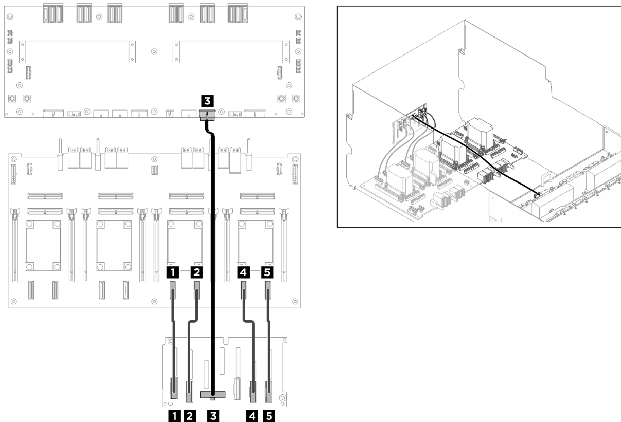
図 203. バックプレーン 2 のケーブル配線
