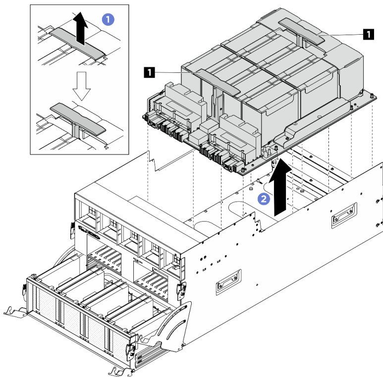
図 128. GPU 複合システムの取り外し
