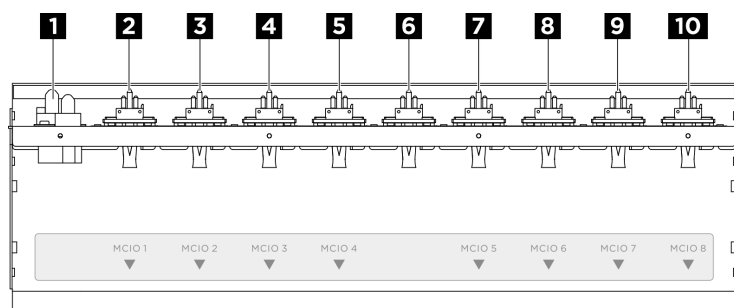
図 187. 前面 PCIe スイッチ・ケーブル・ハーネス・ケーブル
