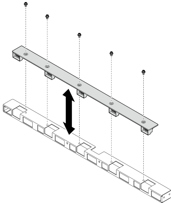
図 38. 前面ファン制御ボードの取り外し
