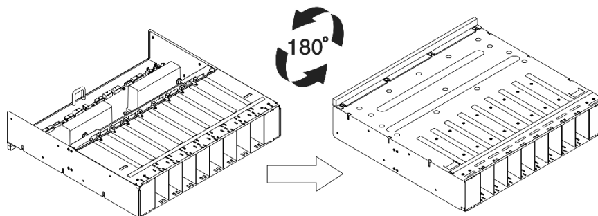
図47. 電源複合システムを上下逆さまにする
