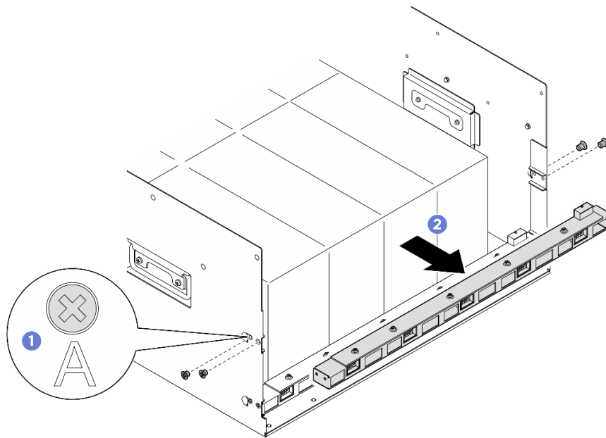
図42. 背面ファン制御ボード・アセンブリの取り外し
