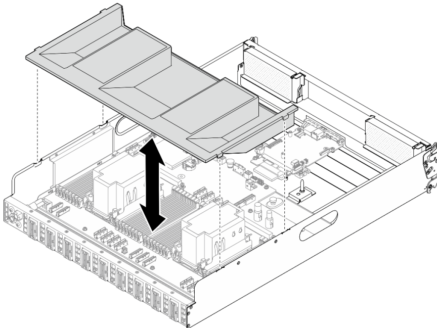
図 81. プロセッサ・エアー・バッフルの取り外し
