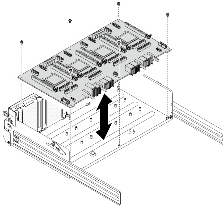
図 152. PCIe スイッチ・ボードの取り付け
