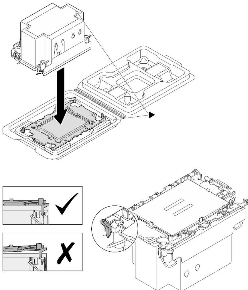
図 93. 配送用トレイのプロセッサーで PHM を取り付けます。
