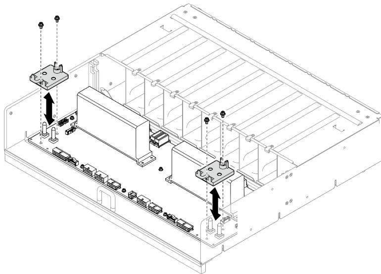
図96. ケーブル保持具の取り外し
