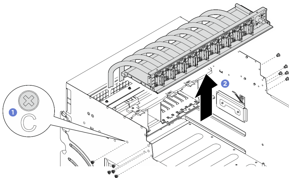
図 163. 前面 PCIe スイッチ・ケーブル・ハーネスの取り外し
