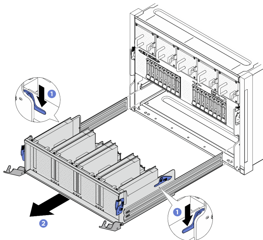
図 179. 8U GPU シャトルからの PCIe スイッチ・シャトルの取り外し
