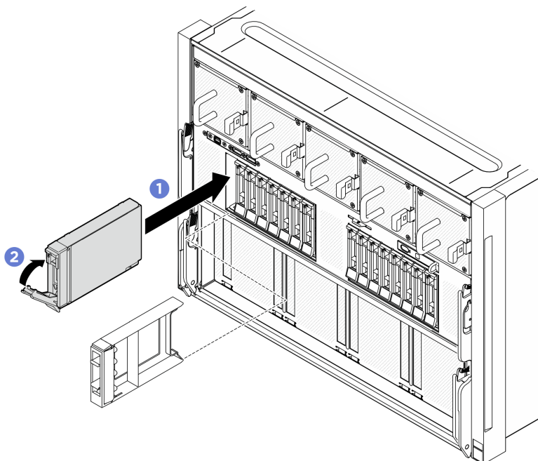
図20. 2.5 型ホット・スワップ・ドライブの取り付け
