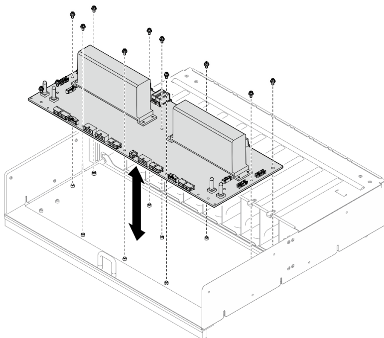
図 74. 分電盤の取り外し
