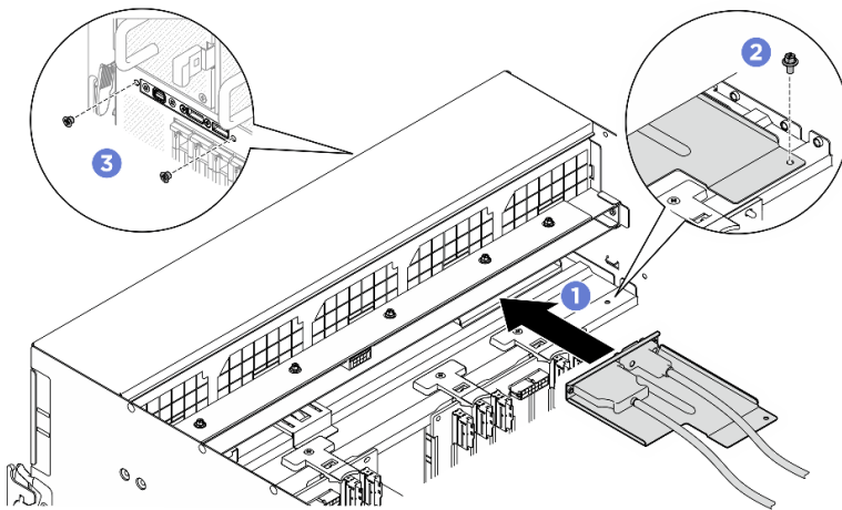
図 171. 前面 I/O モジュールの取り付け
