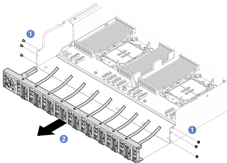
図 172. 背面 PCIe スイッチ・ケーブル・ハーネスの取り外し
