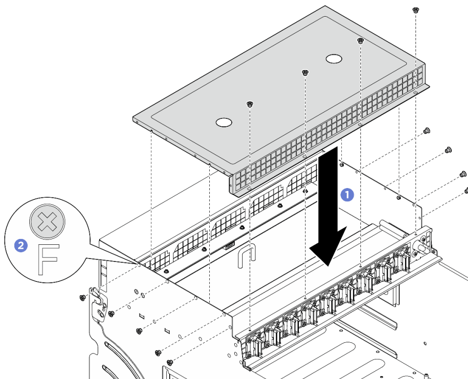
図26. ケーブル・カバーの取り付け
