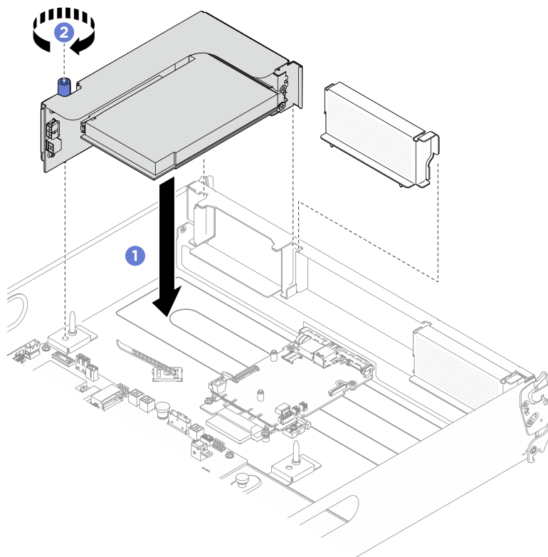
図70. PCIe ライザー・アセンブリーの取り付け
