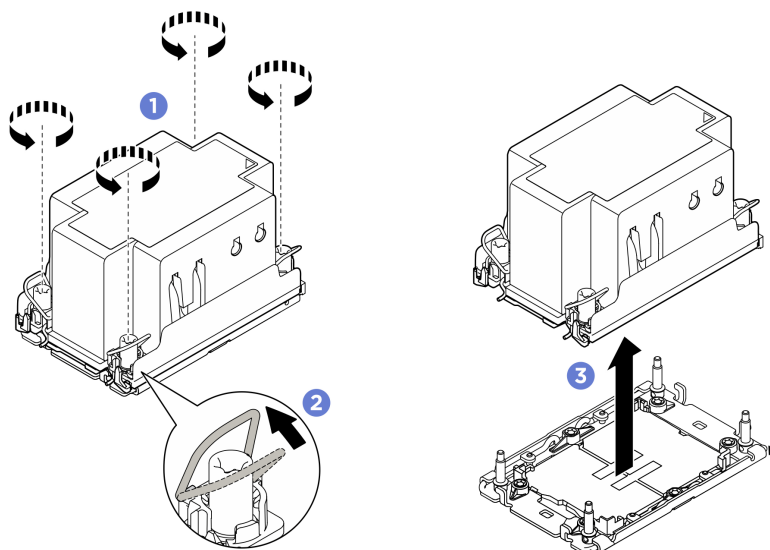
図 87. PHM の取り外し
