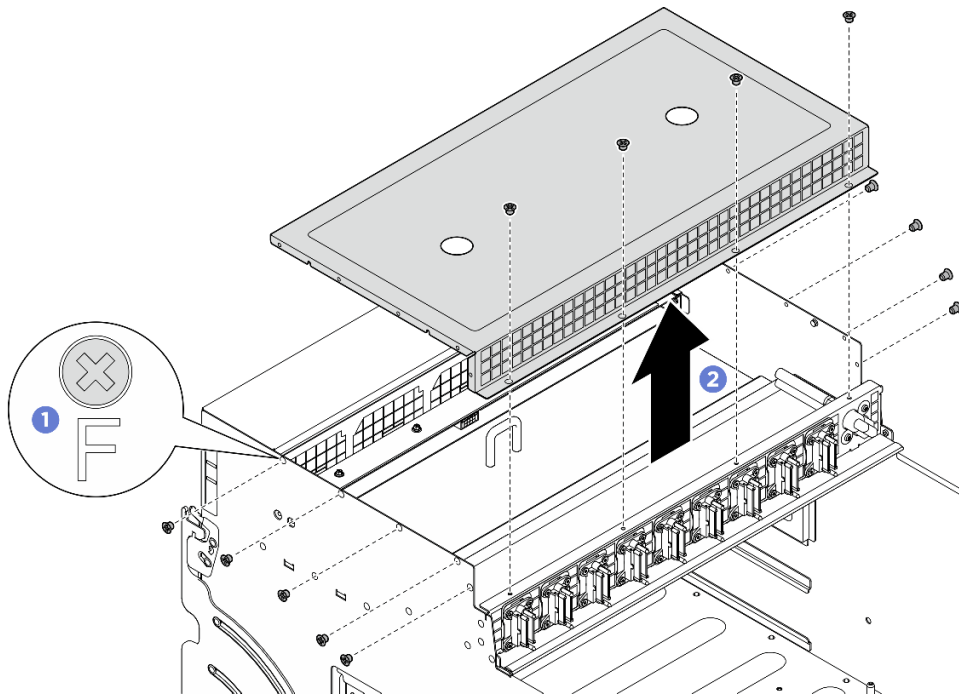
図 25. ケーブル・カバーの取り外し
