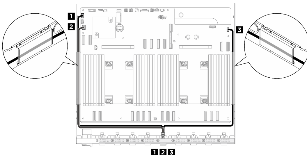
図 197. 前面 I/O モジュールおよび内蔵診断パネルのケーブル配線
