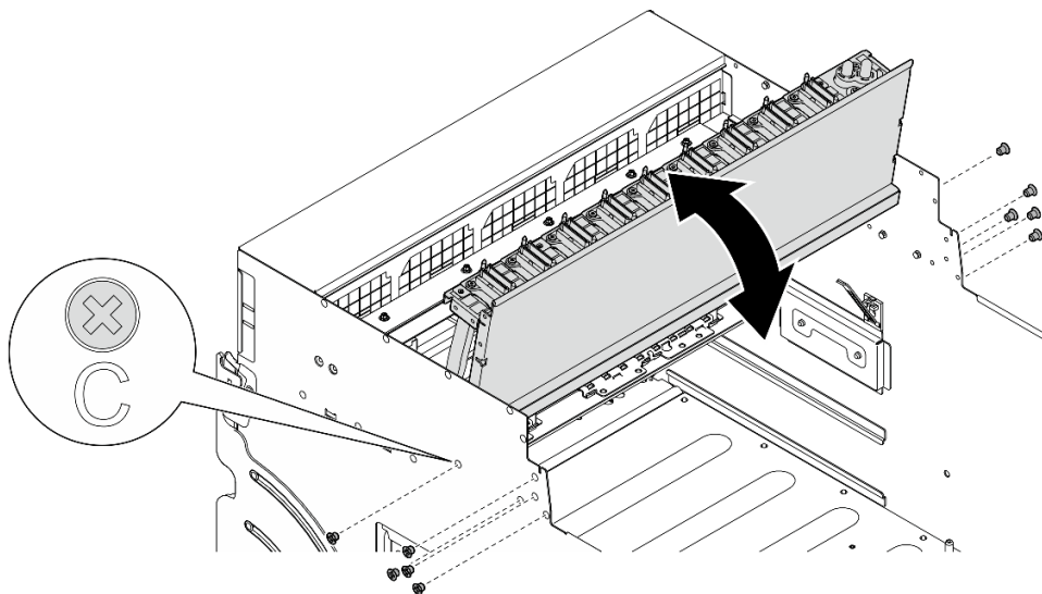
図 132. 前面 PCIe スイッチ・ケーブル・ハーネスをひっくり返す
