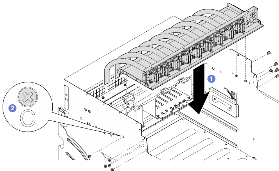
図 169. 前面 PCIe スイッチ・ケーブル・ハーネス の取り付け
