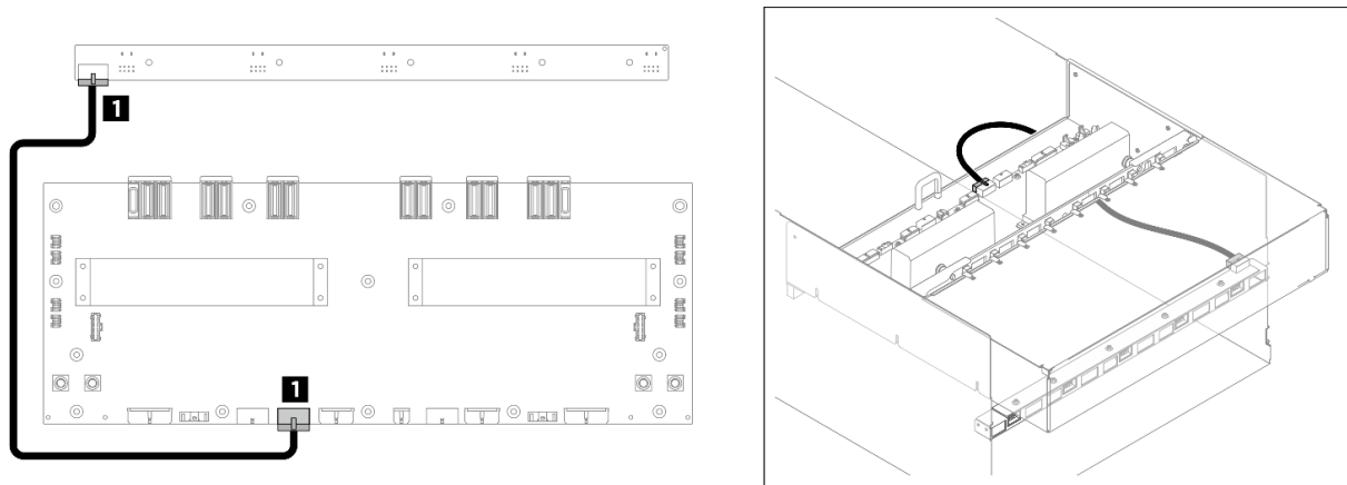
図 195. 背面ファン制御ボード (上部) ケーブル配線
