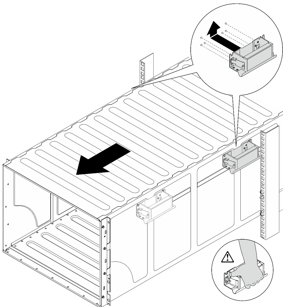
図7. 後部ハンドルの取り付け
