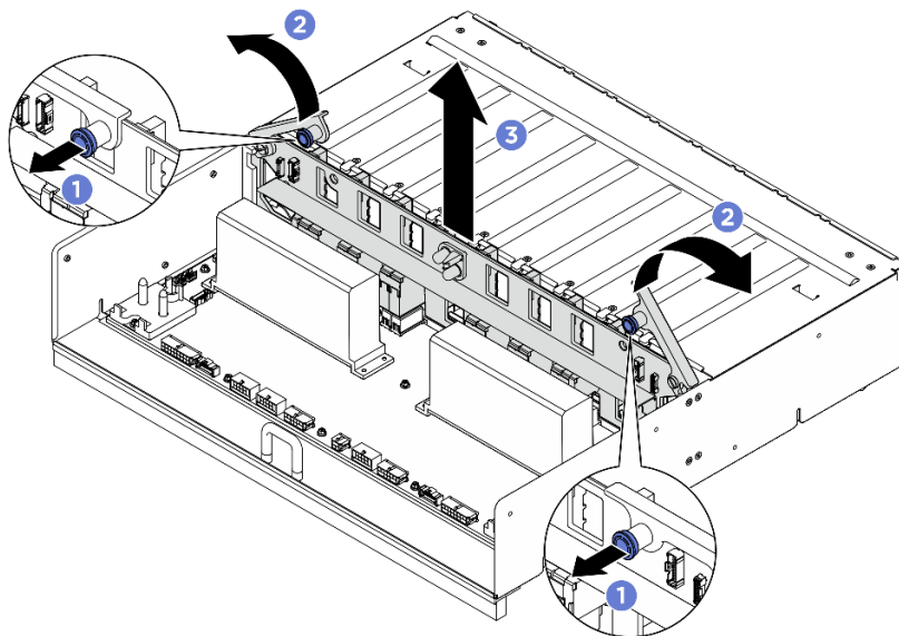
図 101. PSU 変換コネクターの取り外し
