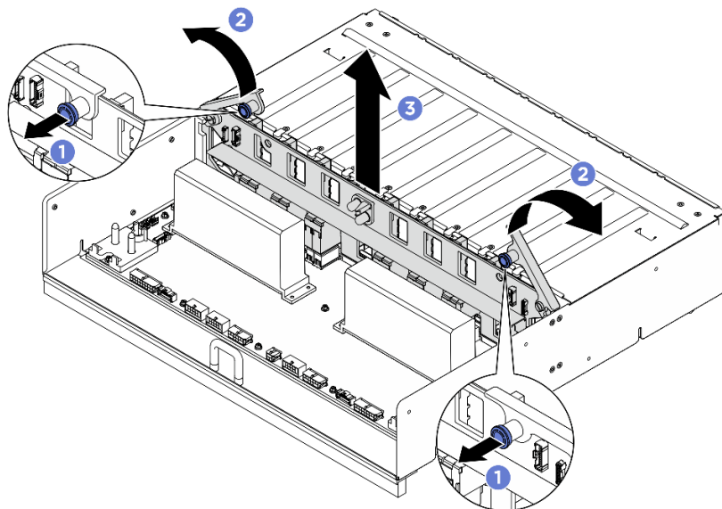
図 95. PSU 変換コネクタの取り外し
