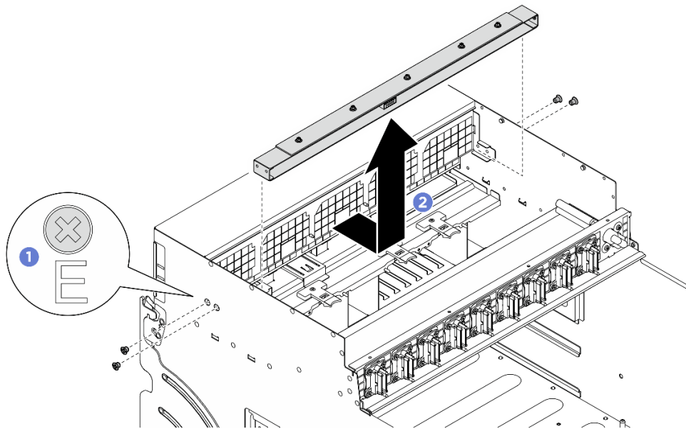
図37. 前面ファン制御ボード・アセンブリーの取り外し
