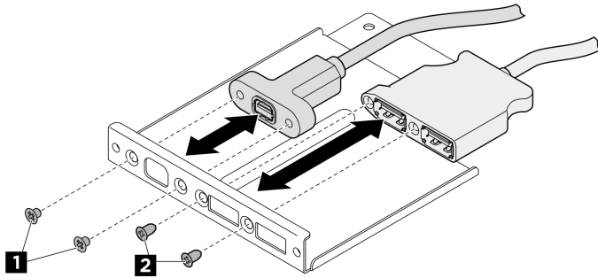
図 170. 前面 I/O モジュール・ケーブルの取り付け
