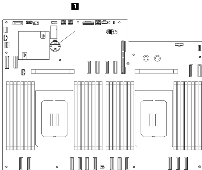
図 27. CMOS バッテリーの位置
