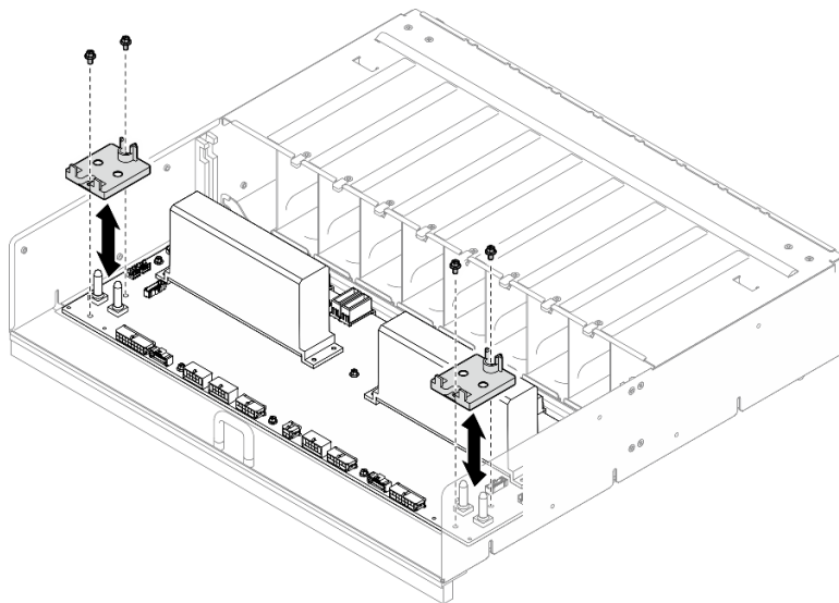
図 76. ケーブル保持具の取り付け
