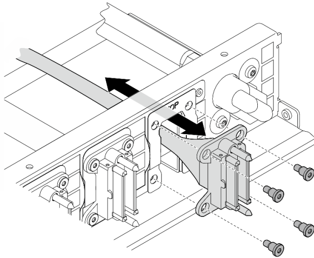
図 164. 前面 I/O モジュール、内蔵診断パネル、GPU 管理、または信号ケーブルの取り外し
