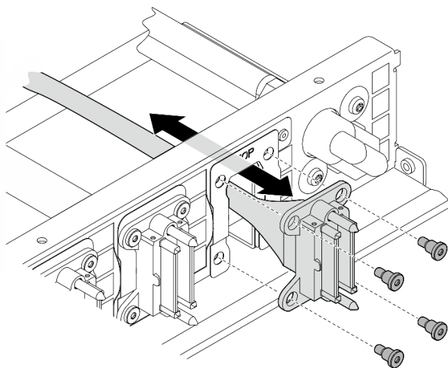
図 167. 前面 I/O モジュール、内蔵診断パネル、GPU 管理、または信号ケーブルの取り付け
