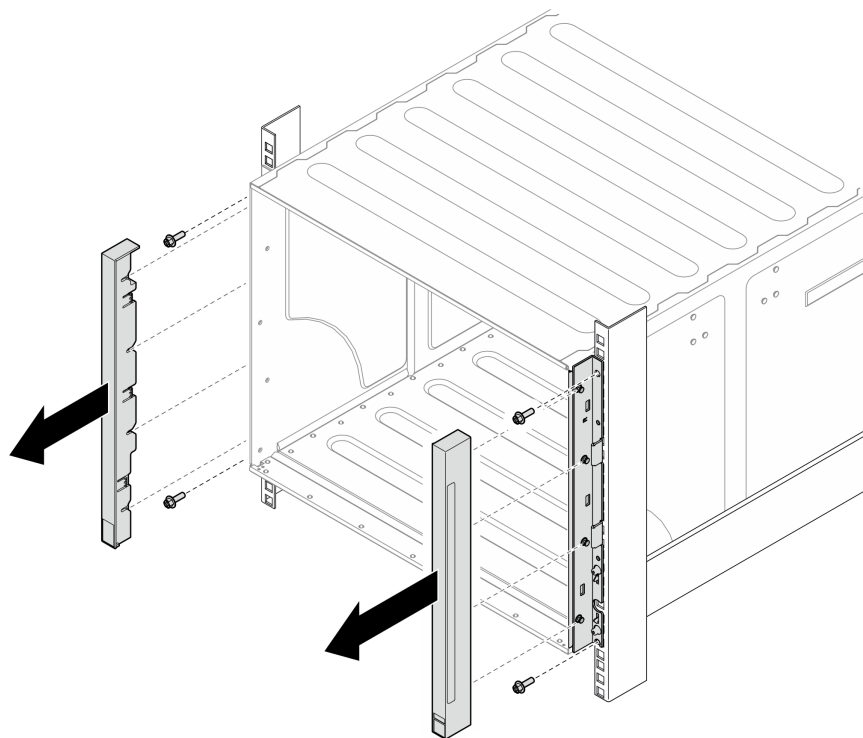
図4. EIA カバーの取り外し
