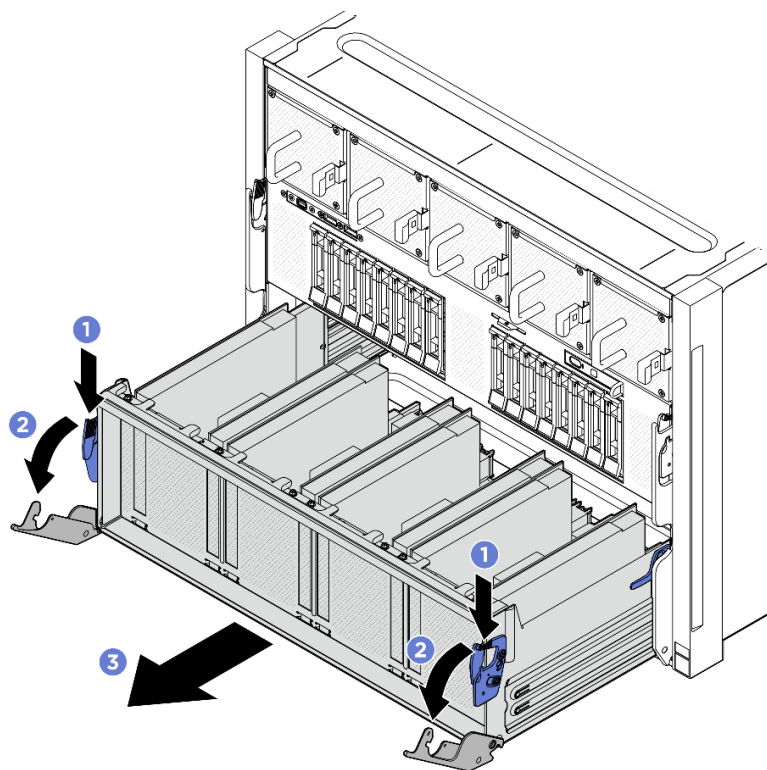
図 116. 停止位置までの PCIe スイッチ・シャトルの取り外し
