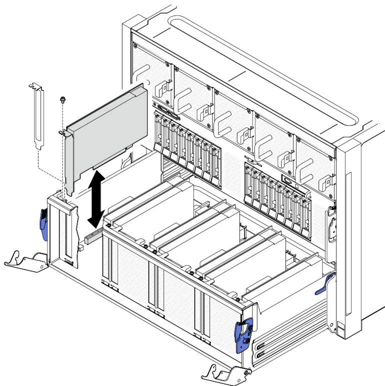
図 156. 前面 PCIe アダプターの取り外し
