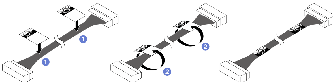
図 113. ラベルの貼り付け
