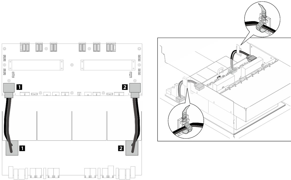
図 205. GPU ベースボードのケーブル配線
