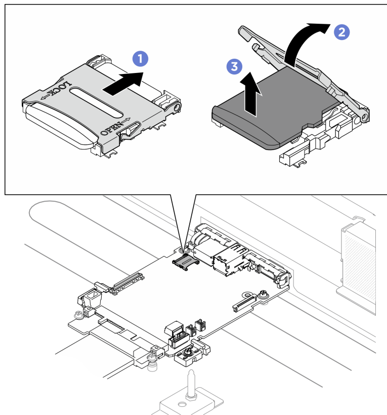
図 62. MicroSD カードの取り外し
