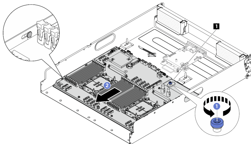
図104. システム・ボードの取り外し
