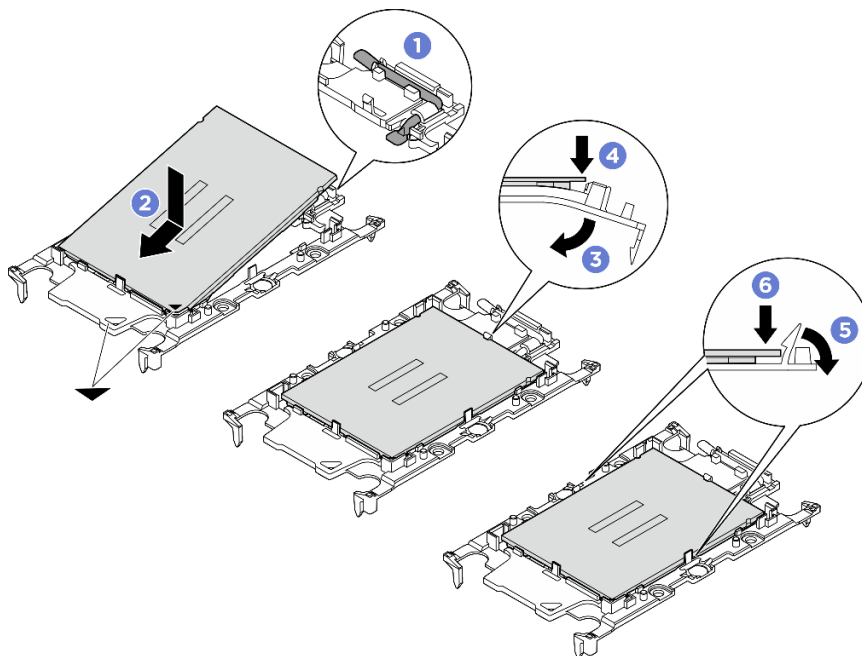
図91. プロセッサ・キャリアの取り付け
