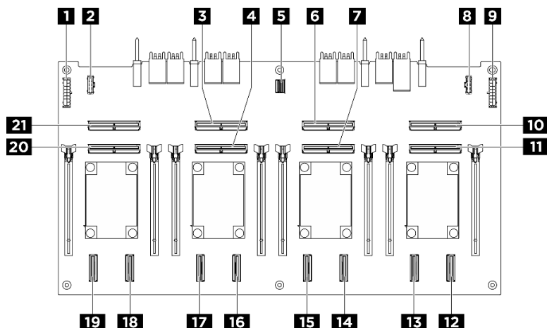
図 186. PCIe スイッチ・ボード コネクタ
