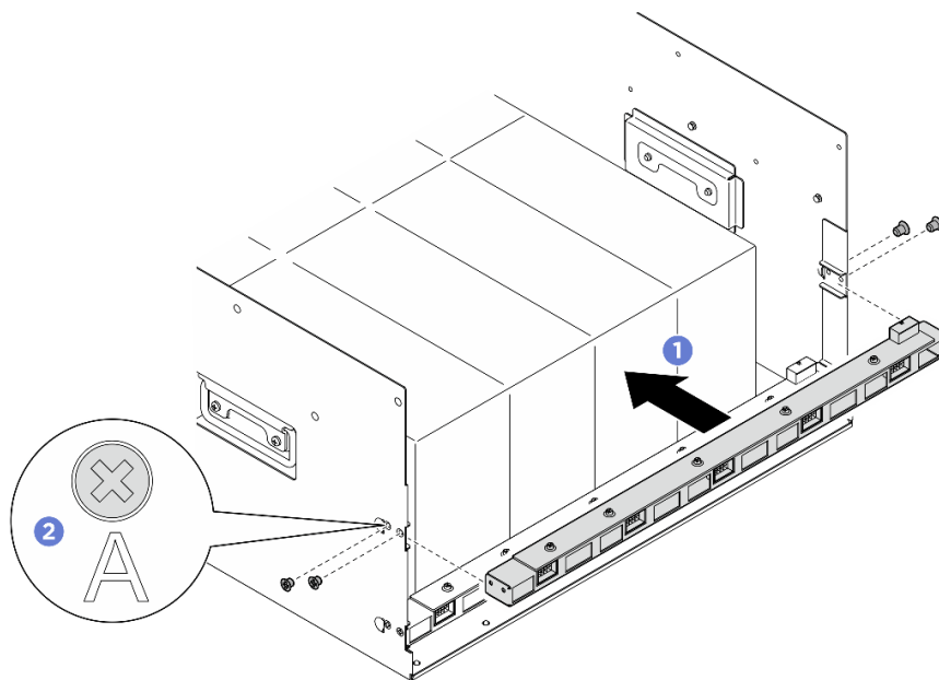
図45. 背面ファン制御ボード・アセンブリーの取り付け
