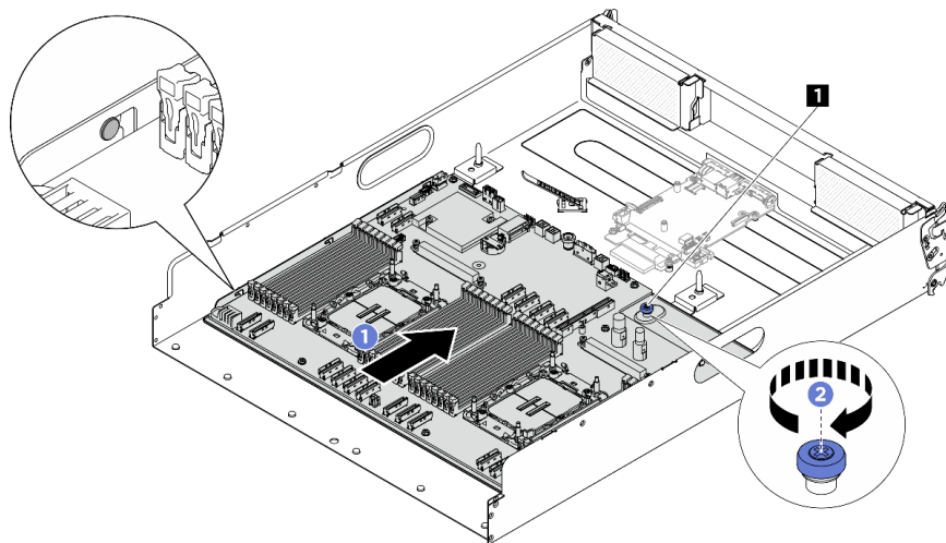
図107. システム・ボードの固定
