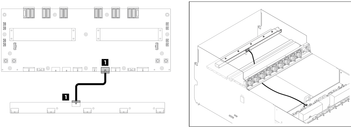
그림 208. 앞면 팬 컨트롤 보드 케이블 배선
