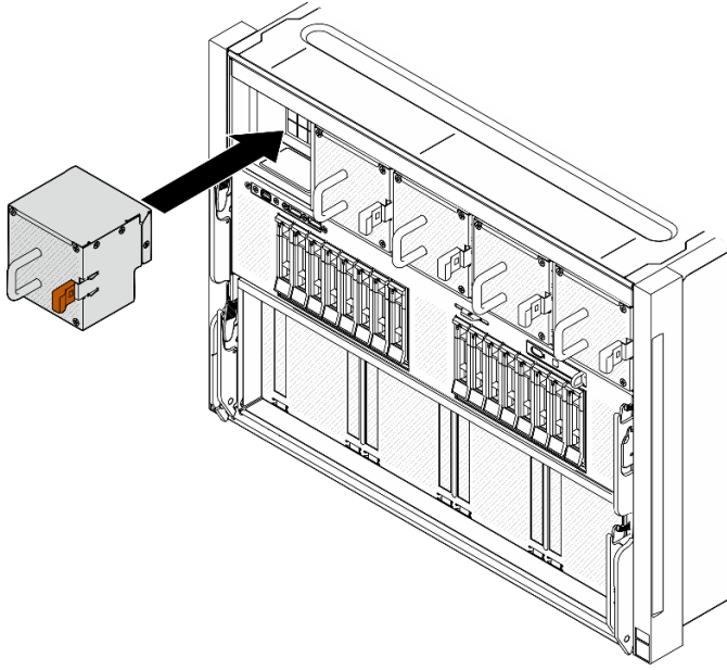
그림 50. 핫 스왑 팬 설치
