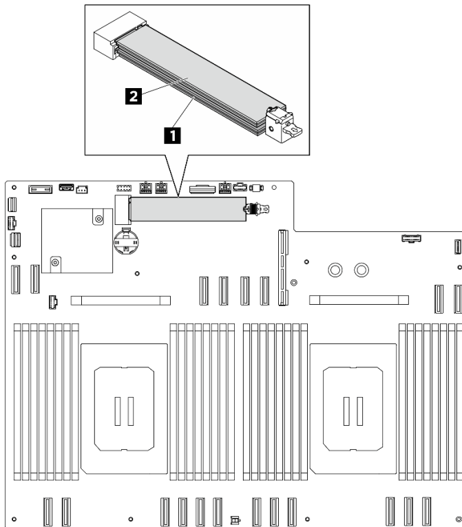
그림 69. M.2 드라이브 슬롯
