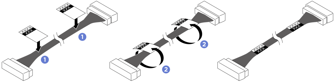
그림 127. 레이블 부착
