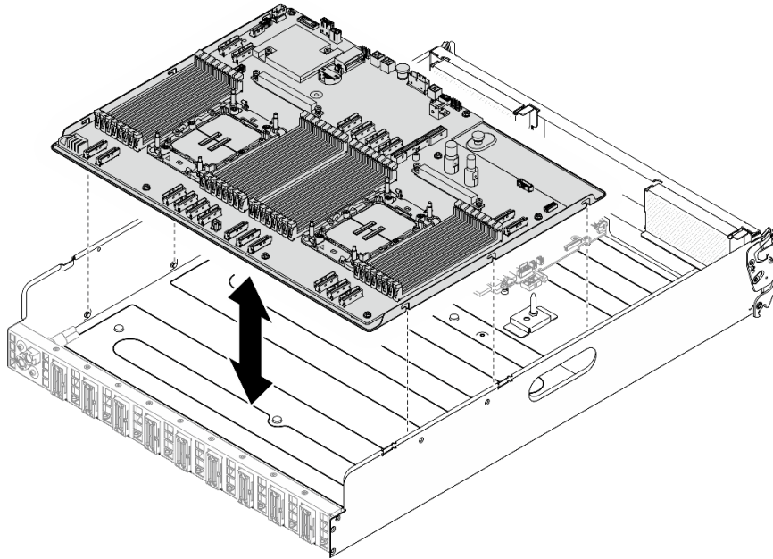
그림 120. 시스템 보드 설치
