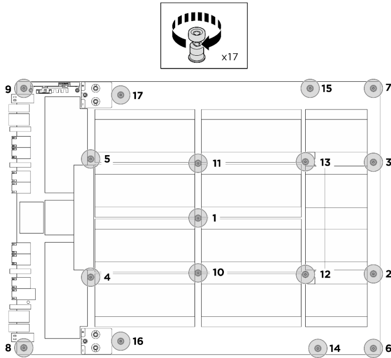
그림 145. 나사 설치
