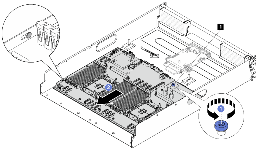
그림 236. 시스템 보드 분리
