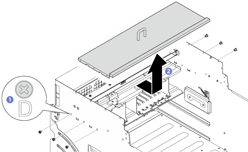
그림 162. I/O 덮개 제거
