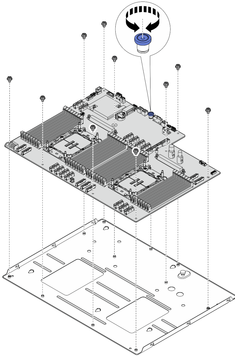
그림 241. 부품 제거
