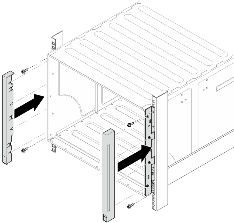
그림 28. EIA 랙개 설치
