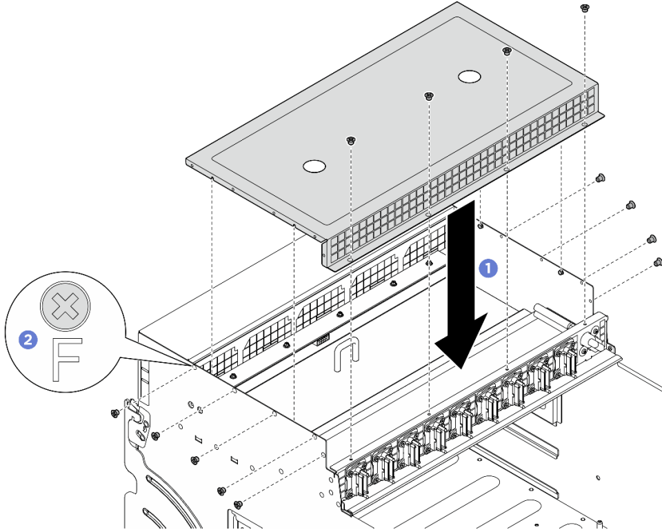
그림 40. 케이블 덮개 설치
