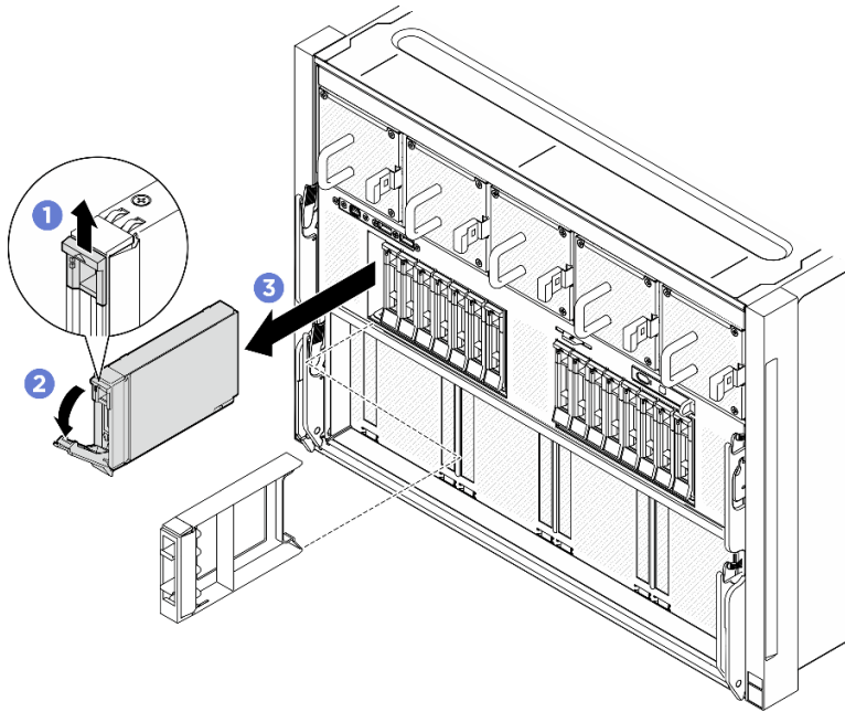
그림 32. 2.5인치 핫 스왑 드라이브 제거
