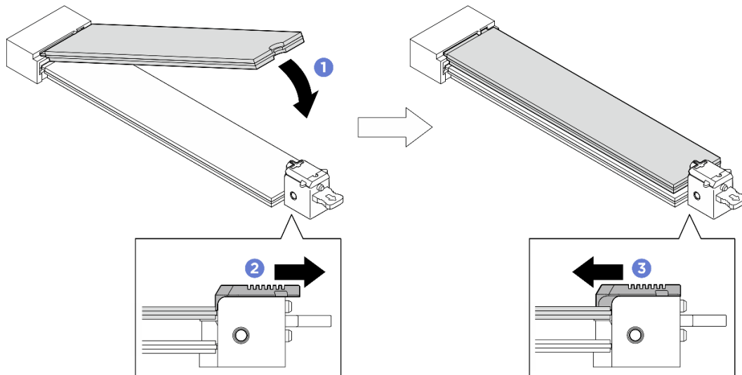
그림 71. 상단 M.2 드라이브 설치
