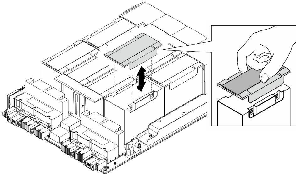
그림 159. 플라스틱 덮개 설치
