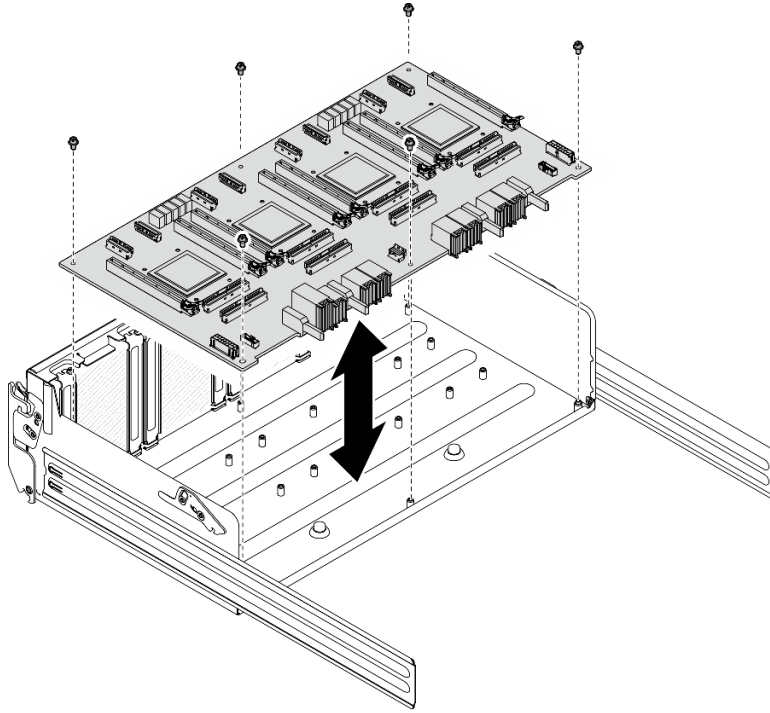
그림 166. PCIe 스위치 보드 설치
