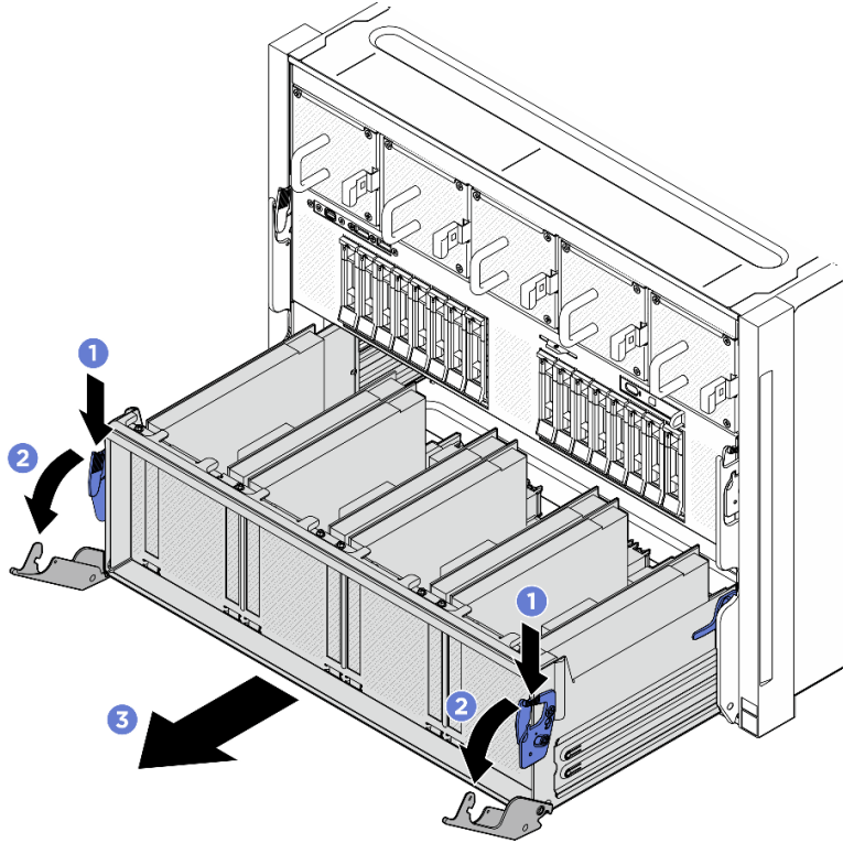
그림 169. 고정 위치까지 PCIe 스위치 셔틀 제거
