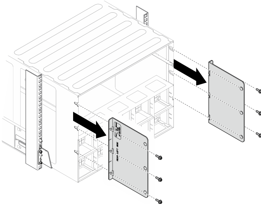
그림 16. 상단 지지 브래킷 제거
