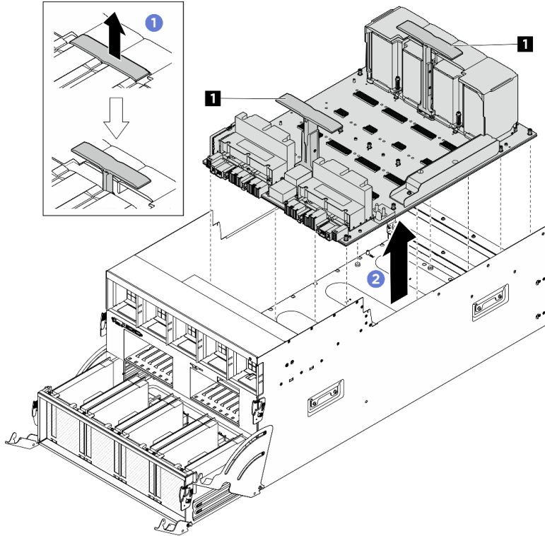
그림 133. GPU 베이스보드 제거
