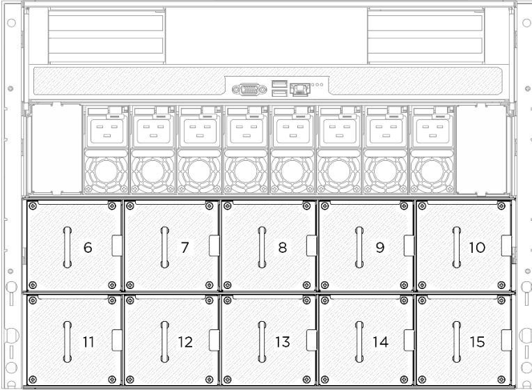
그림 46. 뒷면 팬 번호
