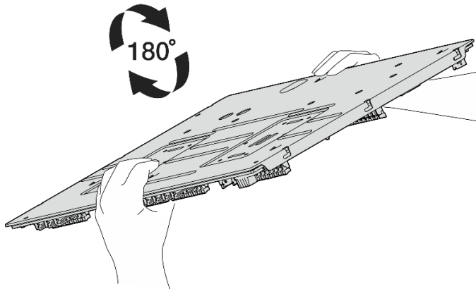
그림 240. 시스템 보드 어셈블리를 올바른 방향으로 돌리기
