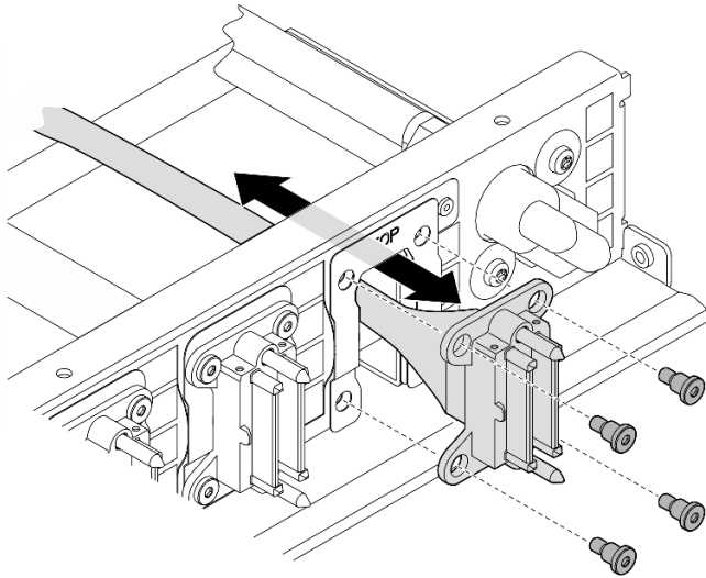
그림 181. 앞면 I/O 모듈, 내장형 진단 패널, GPU 관리 또는 신호 케이블 설치
