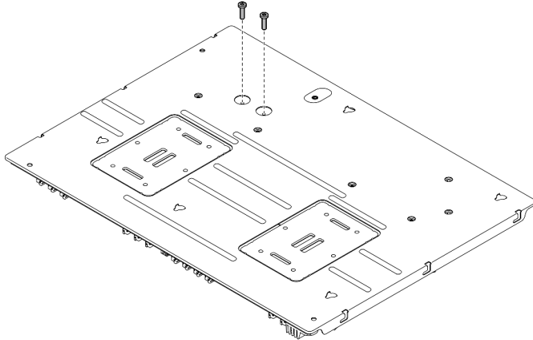
그림 239. 나사 제거
