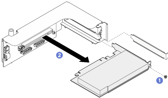
그림 80. 뒷면 PCIe 어댑터 제거
