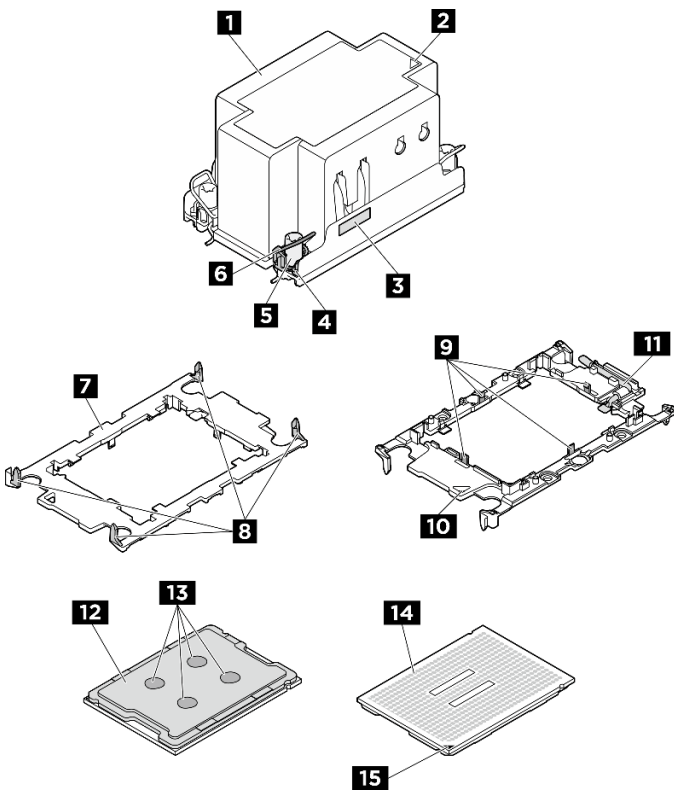
그림 104. PHM 구성 요소
