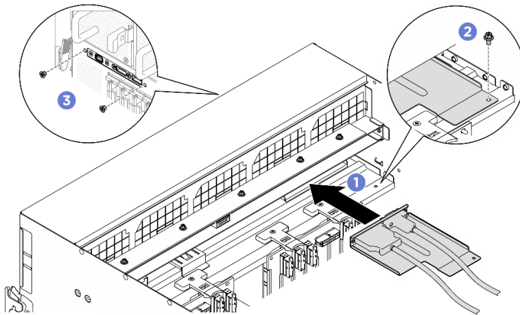
그림 185. 앞면 I/O 모듈 설치
