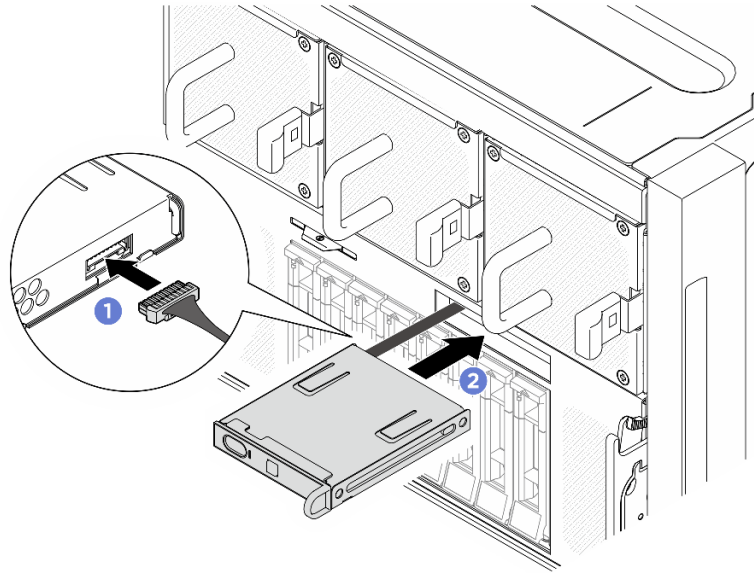
그림 65. 내장형 진단 패널 설치
