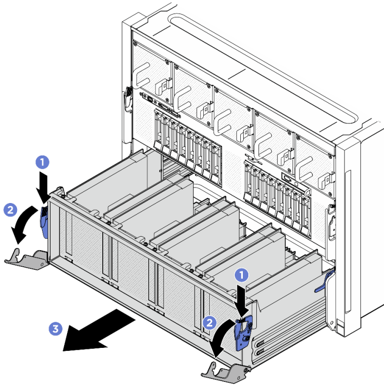
그림 130. 고정 위치까지 PCIe 스위치 셔틀 제거
