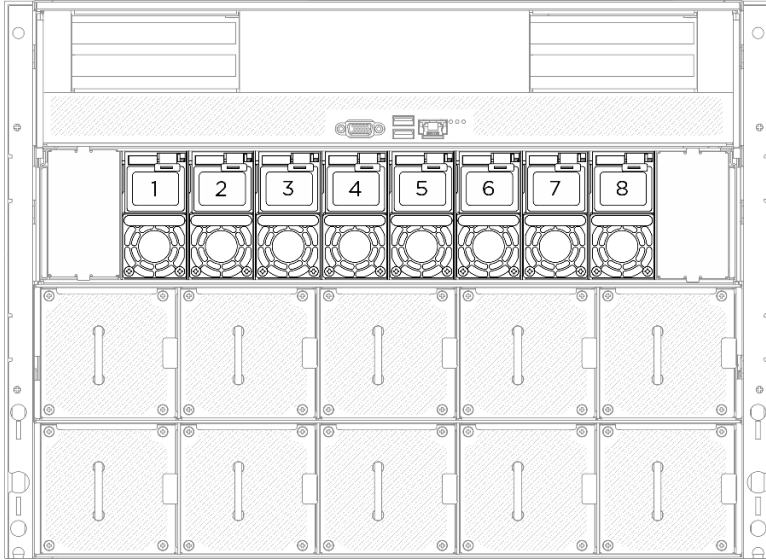
그림 93. 전원 공급 장치 베이 번호
