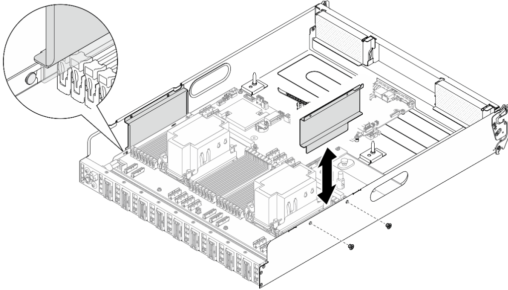
그림 235. 케이블 가이드 제거
