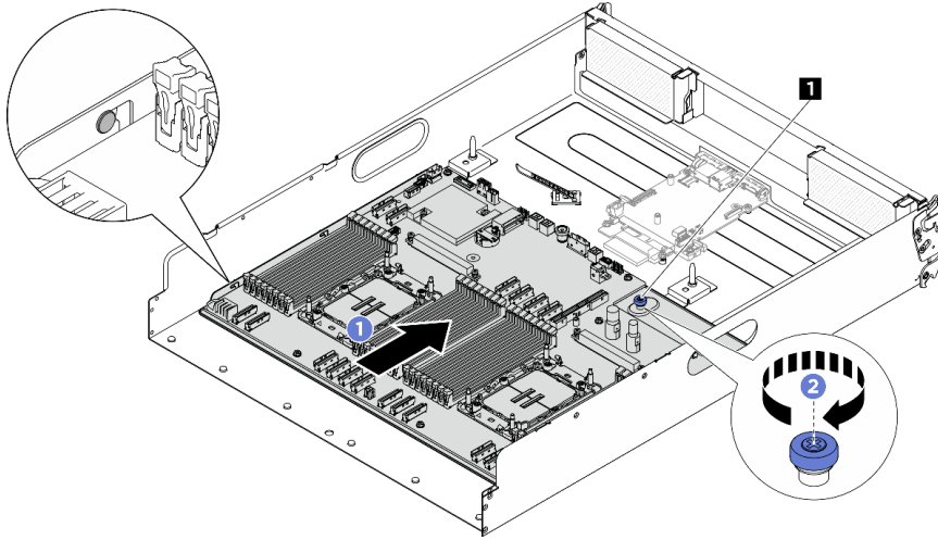
그림 121. 시스템 보드 고정
