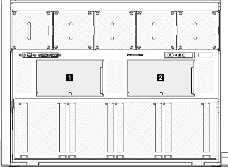
그림 123. 2.5인치 드라이브 백플레인 넘버링
