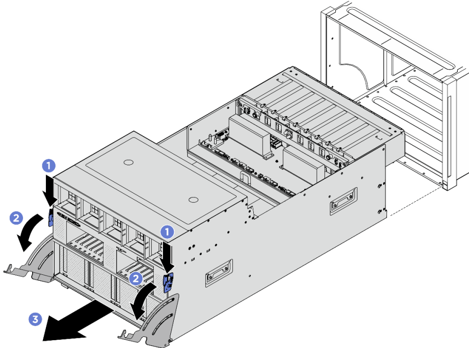
그림 37. 8U GPU 서버 제거
