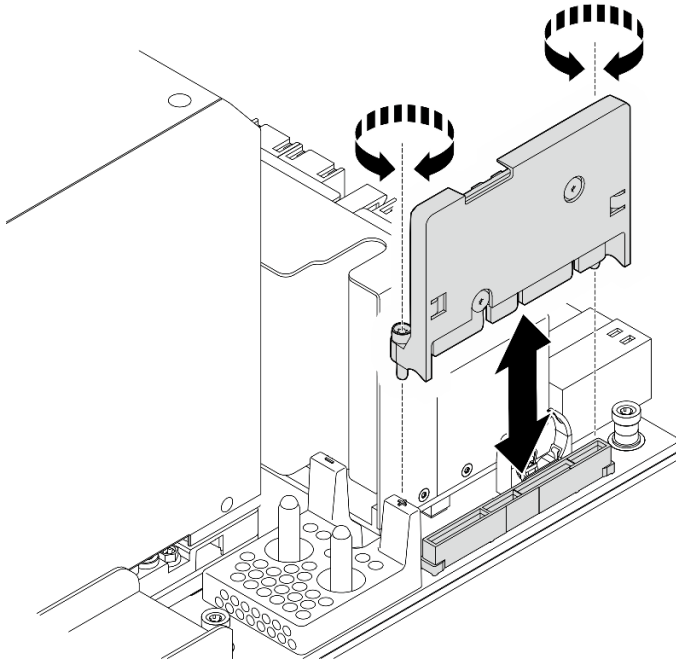
그림 161. HMC 카드 설치
