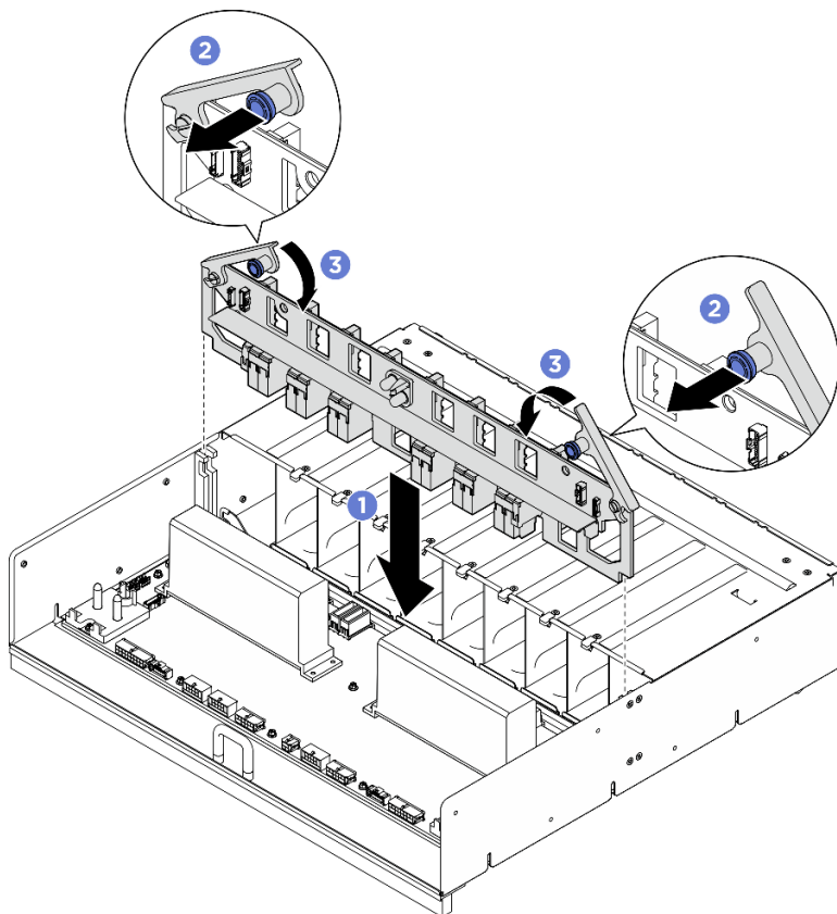
그림 116. PSU 인터포저 설치
