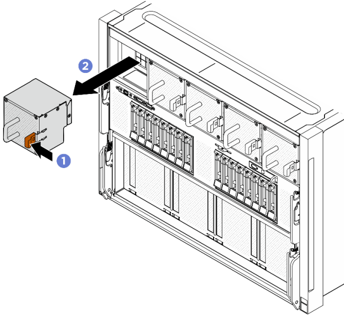
그림 47. 핫 스왑 팬 제거
