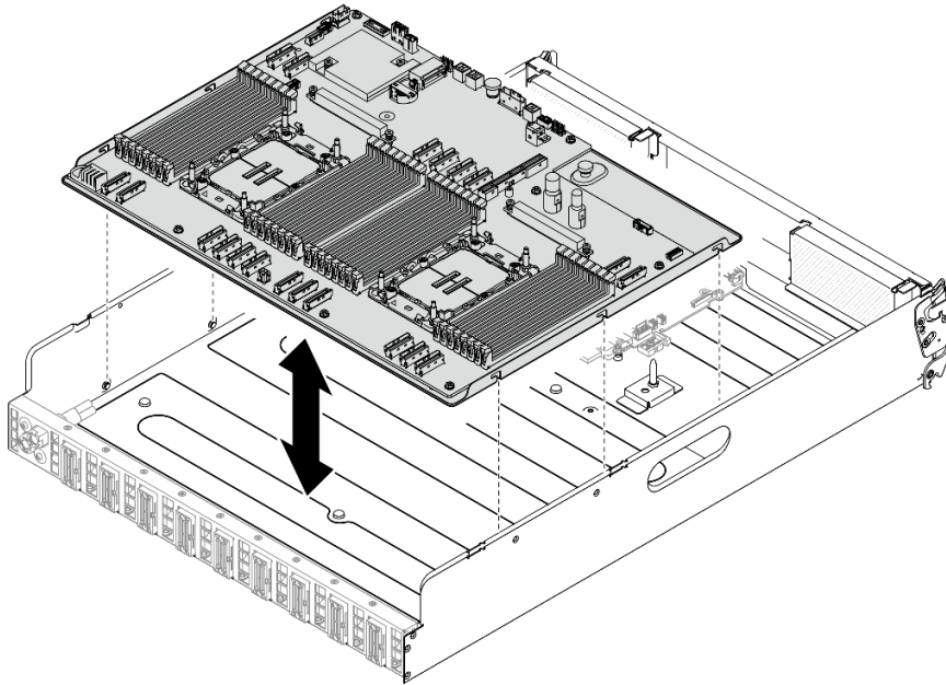
그림 237. 시스템 보드 제거
