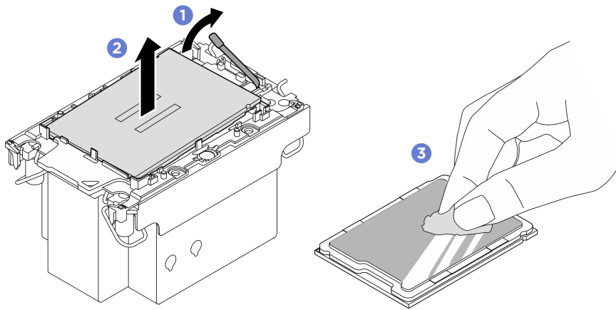
그림 102. 방열판 및 캐리어에서 프로세서 분리 중
