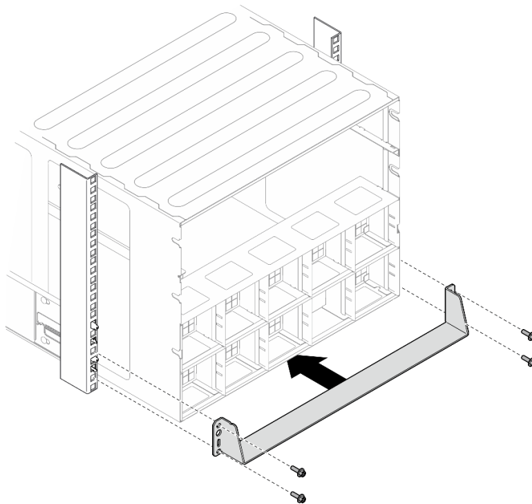
그림 29. 하단 지지 브래킷 설치
