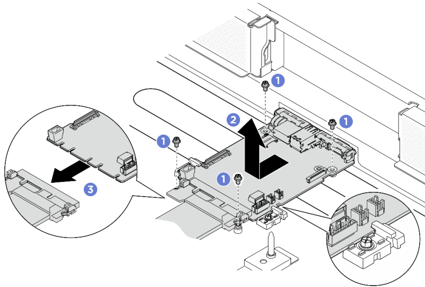
그림 97. 시스템 I/O 보드 제거
