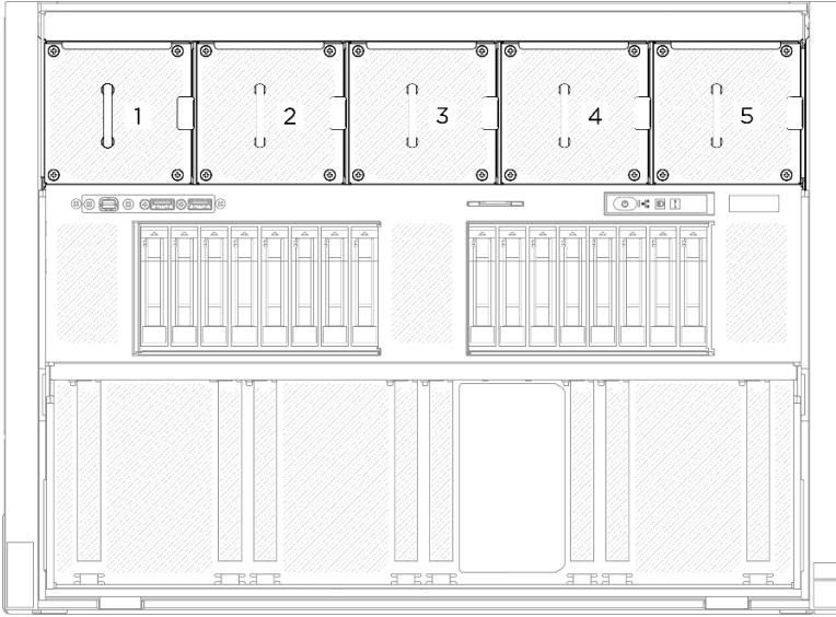
그림 45. 앞면 팬 번호
