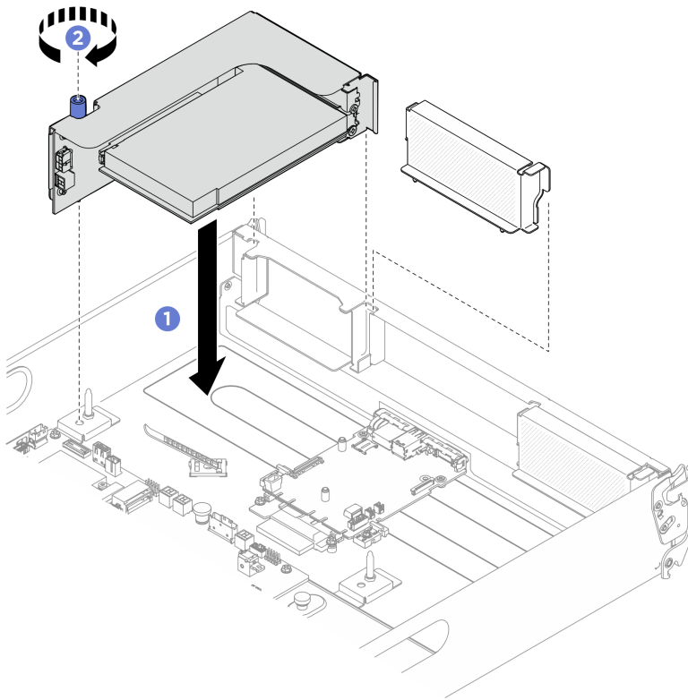
그림 84. PCIe 라이저 어셈블리 설치
