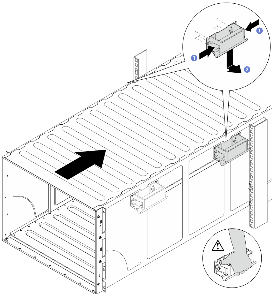
그림 25. 뒷면 손잡이 제거
