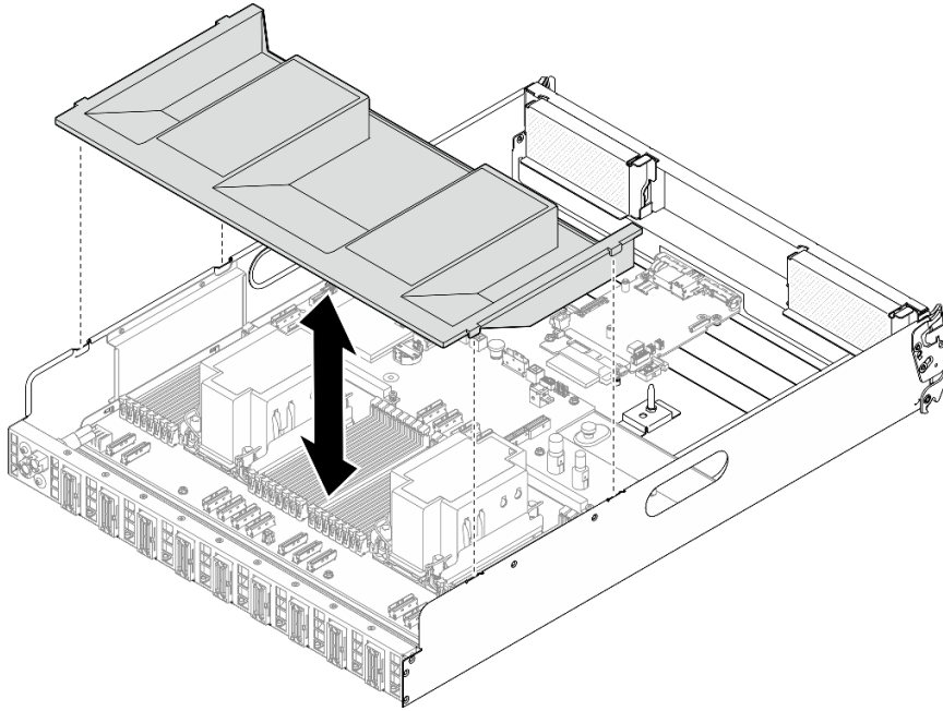
그림 96. 프로세서 공기 조절 장치 설치
