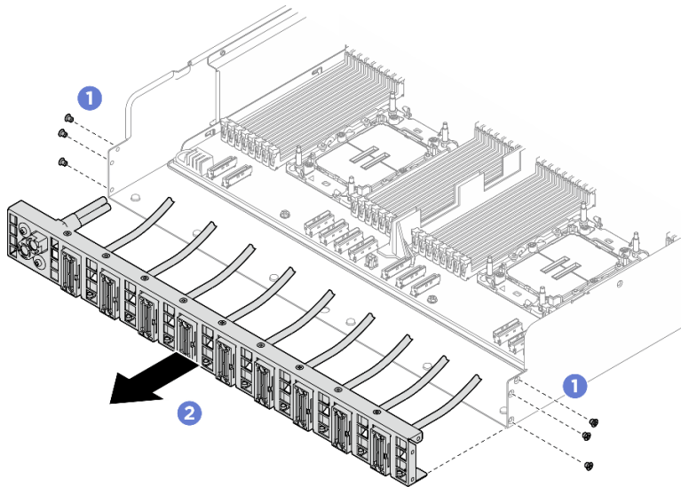
그림 186. 뒷면 PCIe 스위치 케이블 하네스 제거
