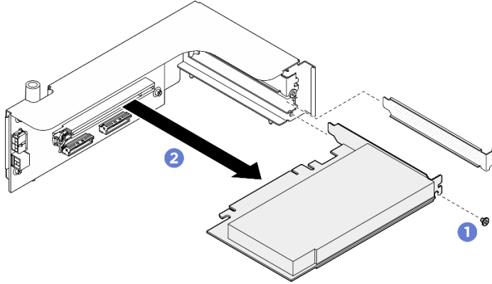
그림 173. 뒷면 PCIe 어댑터 제거
