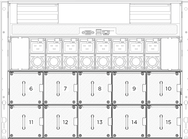
그림 49. 뒷면 팬 번호
