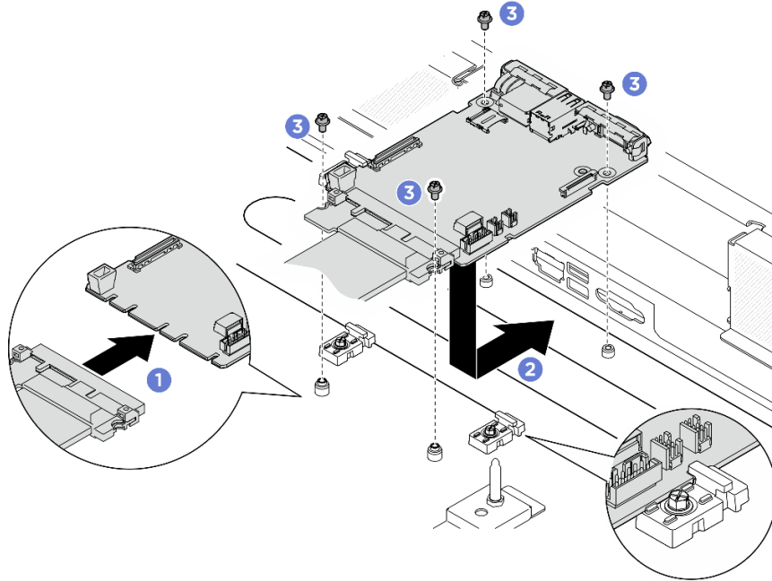
그림 98. 시스템 I/O 보드 설치
