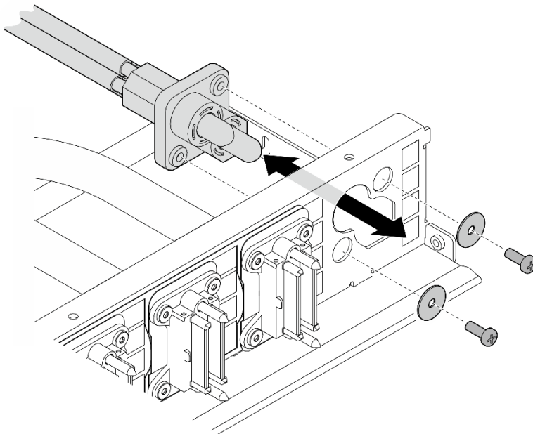
그림 179. 전원 케이블 제거
