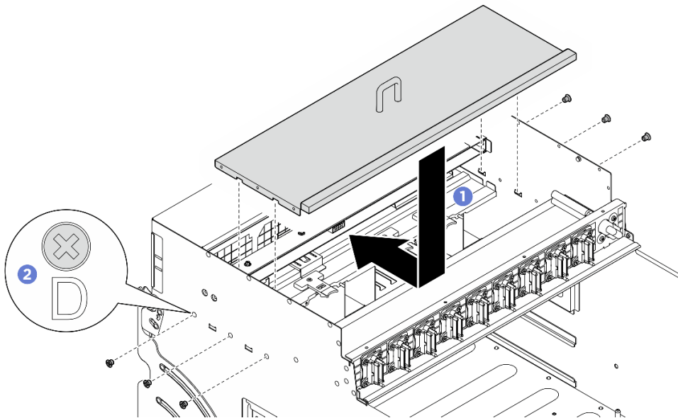
그림 163. I/O 덮개 설치
