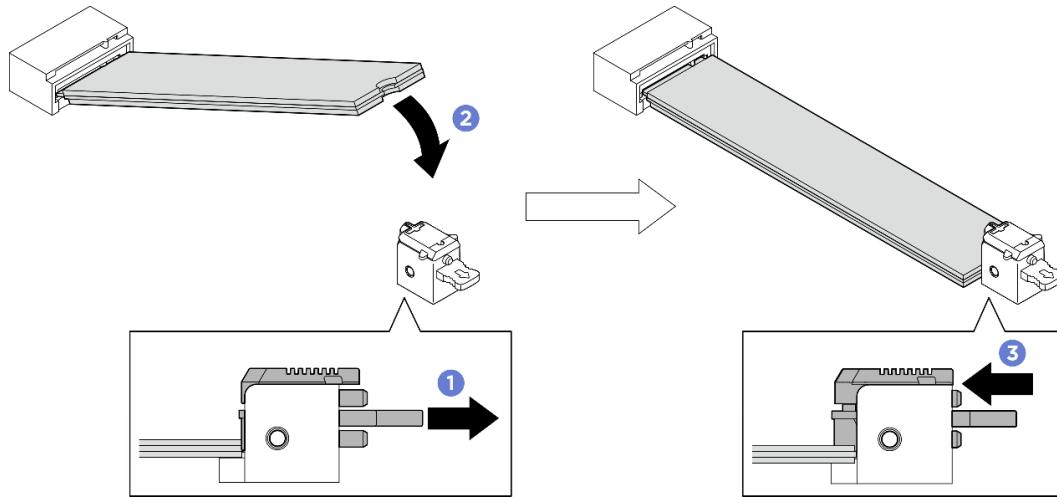
그림 70. 하단 M.2 드라이브 설치
