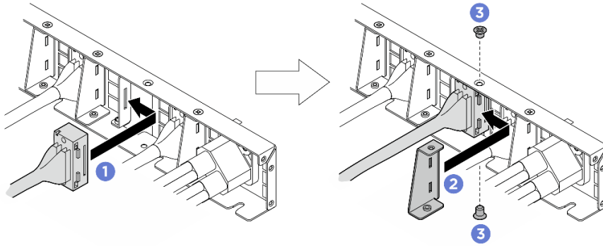
그림 189. 앞면 I/O 모듈, 내장형 진단 패널, GPU 관리 또는 신호 케이블 설치
