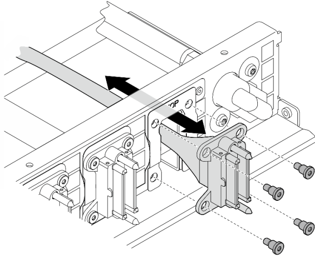
그림 178. 앞면 I/O 모듈, 내장형 진단 패널, GPU 관리 또는 신호 케이블 제거
