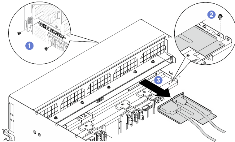
그림 175. 앞면 I/O 모듈 제거
