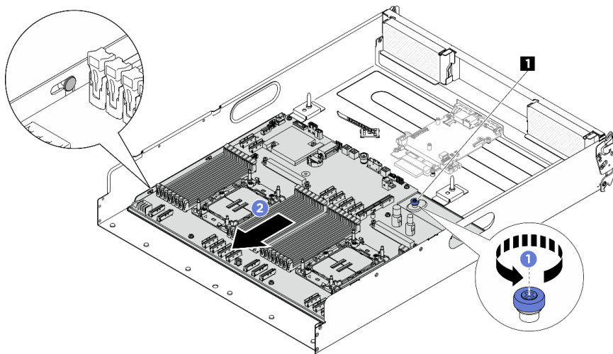
그림 118. 시스템 보드 분리
