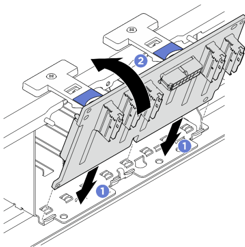
그림 126. 2.5인치 드라이브 백플레인 설치
