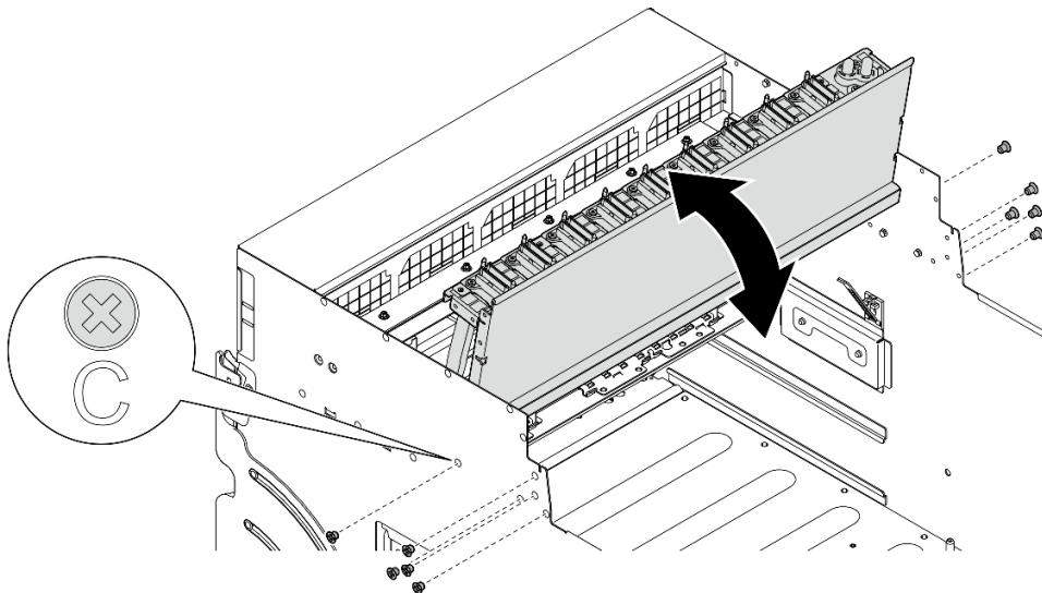
그림 137. 앞면 PCIe 스위치 케이블 하네스 뒤집기
