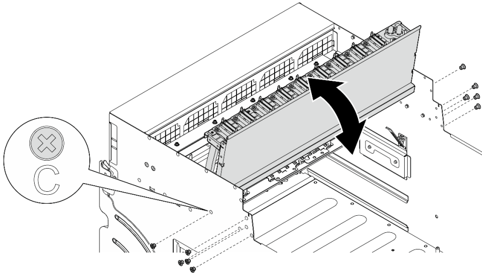
그림 131. 앞면 PCIe 스위치 케이블 하네스 뒤집기
