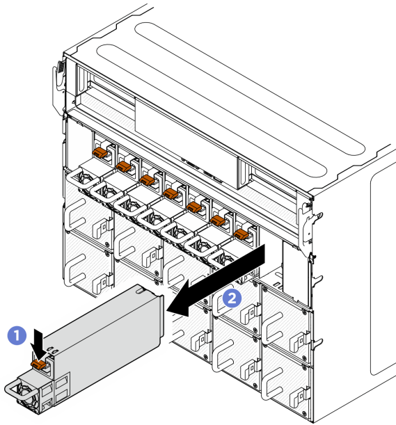
그림 92. 전원 공급 장치 유닛 제거
