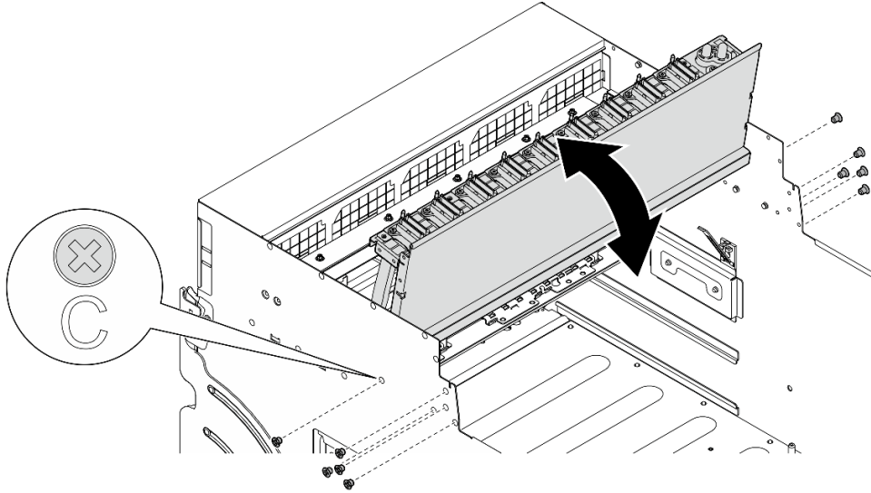
그림 140. 앞면 PCIe 스위치 케이블 하네스 뒤집기
