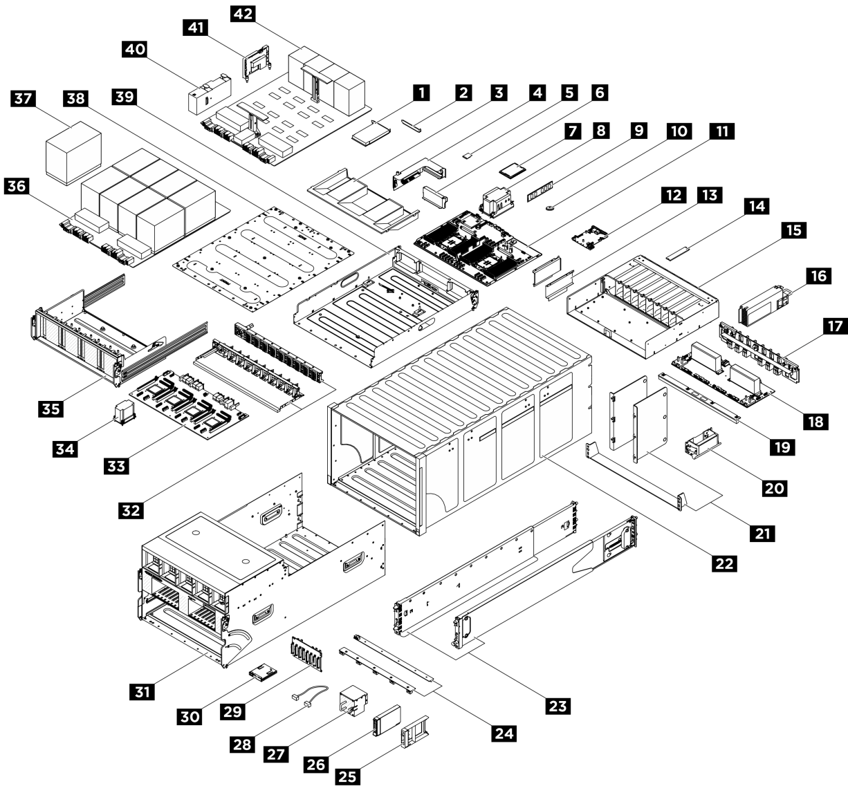
그림 11. 서버 구성 요소
