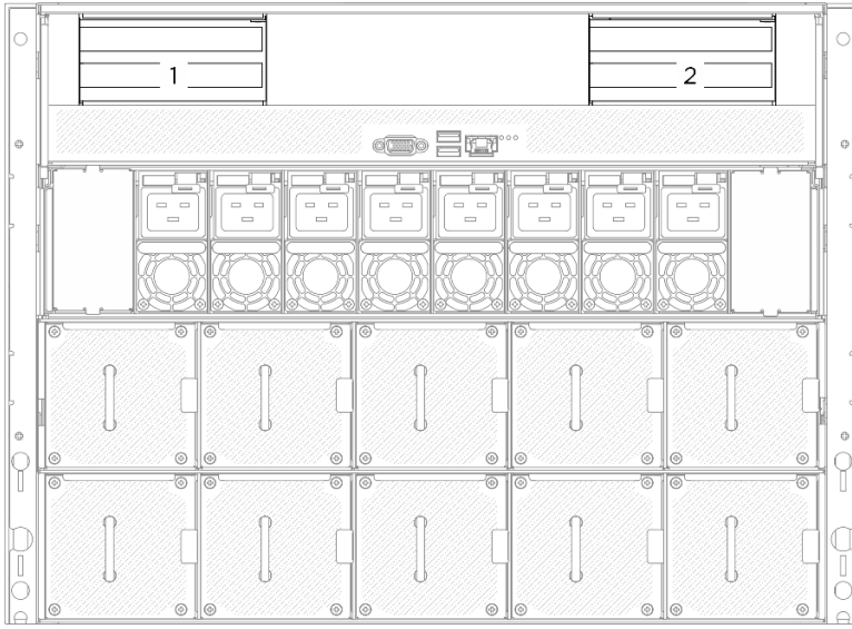
그림 78. PCIe 라이저 위치
