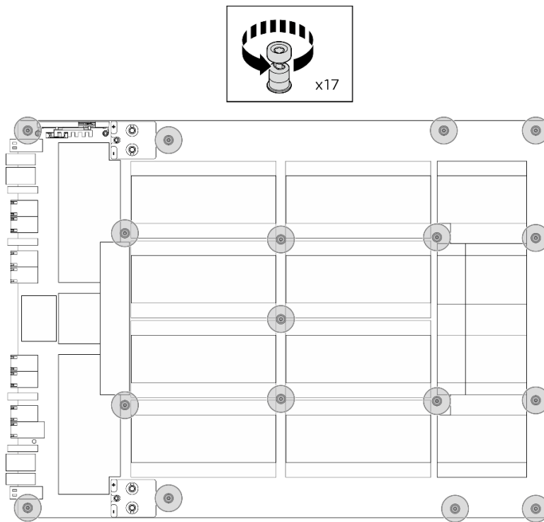
그림 141. 나사 제거
