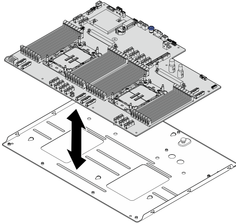
그림 242. 시스템 보드 어셈블리 분해
