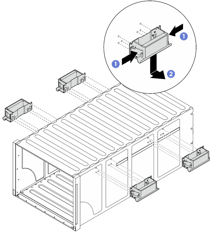
그림 22. 손잡이 제거
