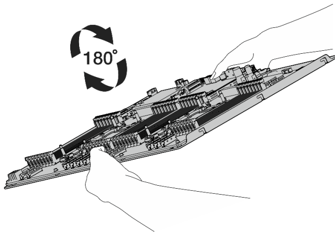
그림 238. 시스템 보드 어셈블리 거꾸로 뒤집기
