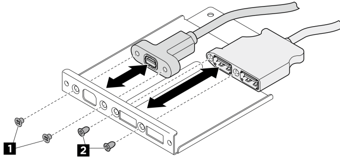
그림 184. 앞면 I/O 모듈 케이블 설치
