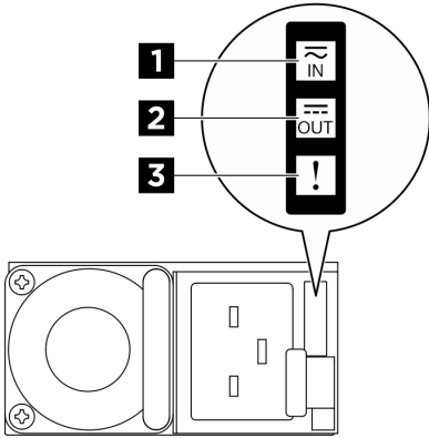
그림 231. CFFv4 전원 공급 장치 LED
