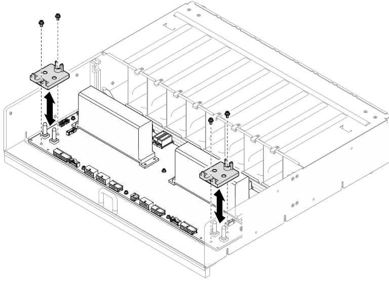
그림 113. 케이블 고정장치 설치
