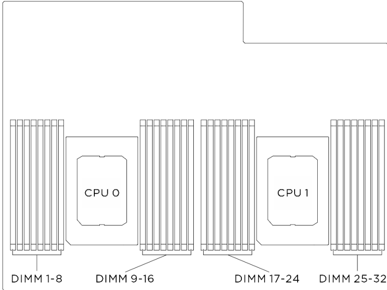
그림 15. 메모리 모듈 및 프로세서 레이아웃
