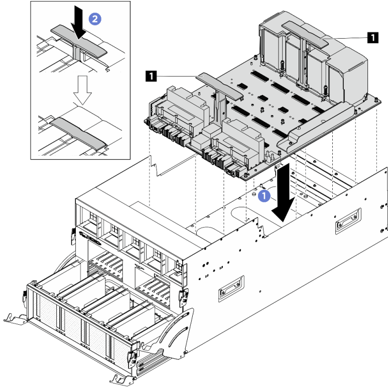
그림 135. GPU 베이스보드 설치
