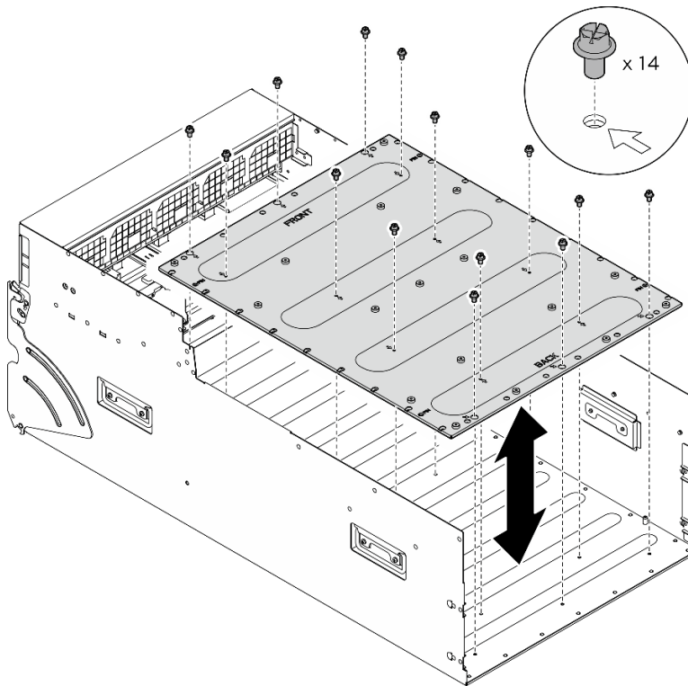
그림 150. GPU 복합체 어댑터판 제거
