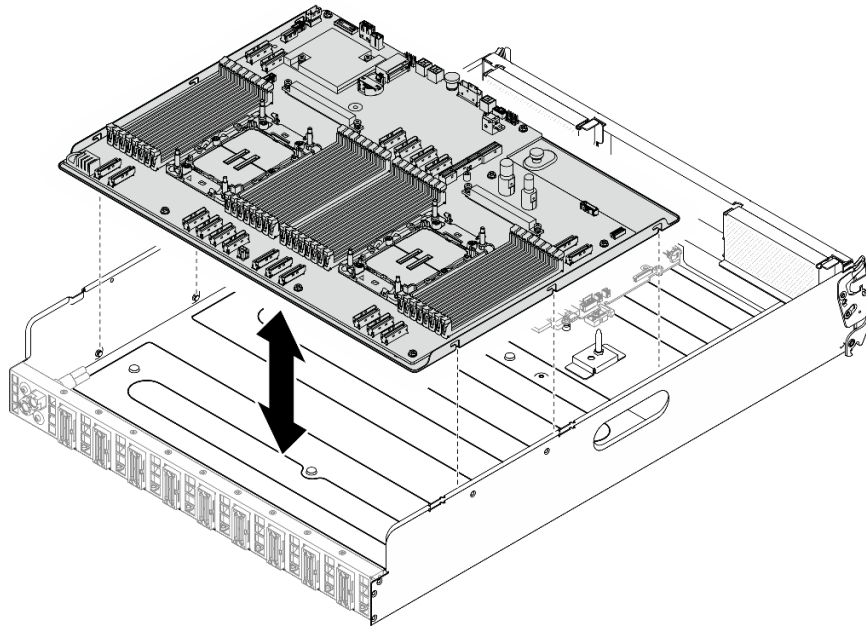
그림 119. 시스템 보드 제거
