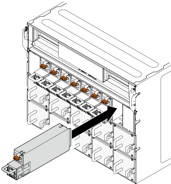
그림 94. 전원 공급 장치 설치
