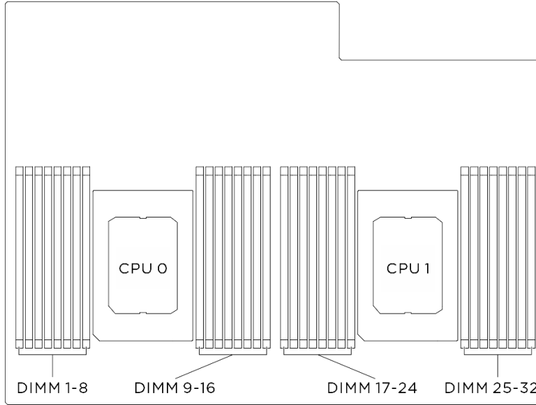
그림 72. 메모리 모듈 및 프로세서 레이아웃
