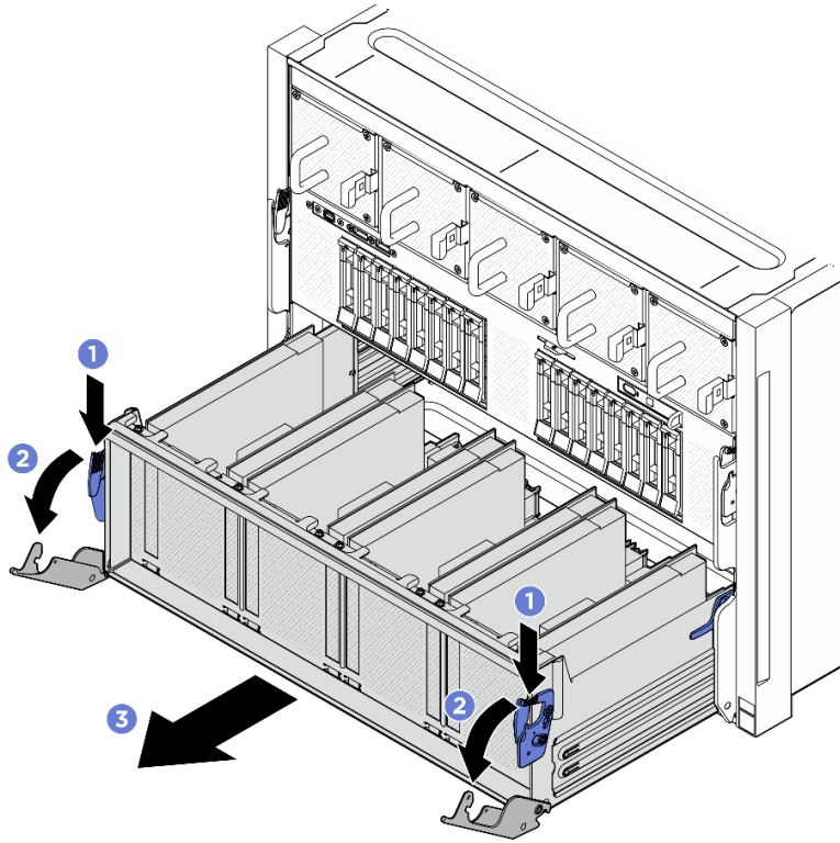
그림 148. 고정 위치까지 PCIe 스위치 셔틀 제거
