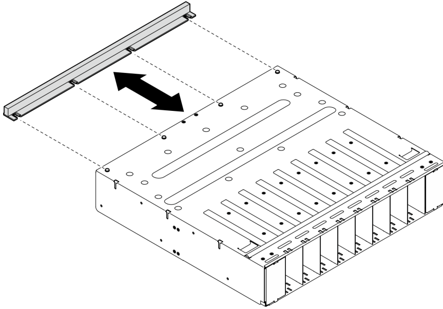
그림 62. GPU 공기 조절 장치 제거
