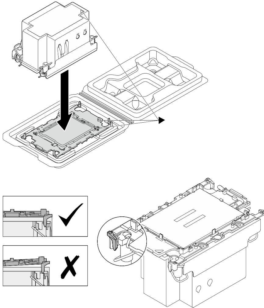
그림 107. 운송 트레이 내 프로세서로 PHM 조립
