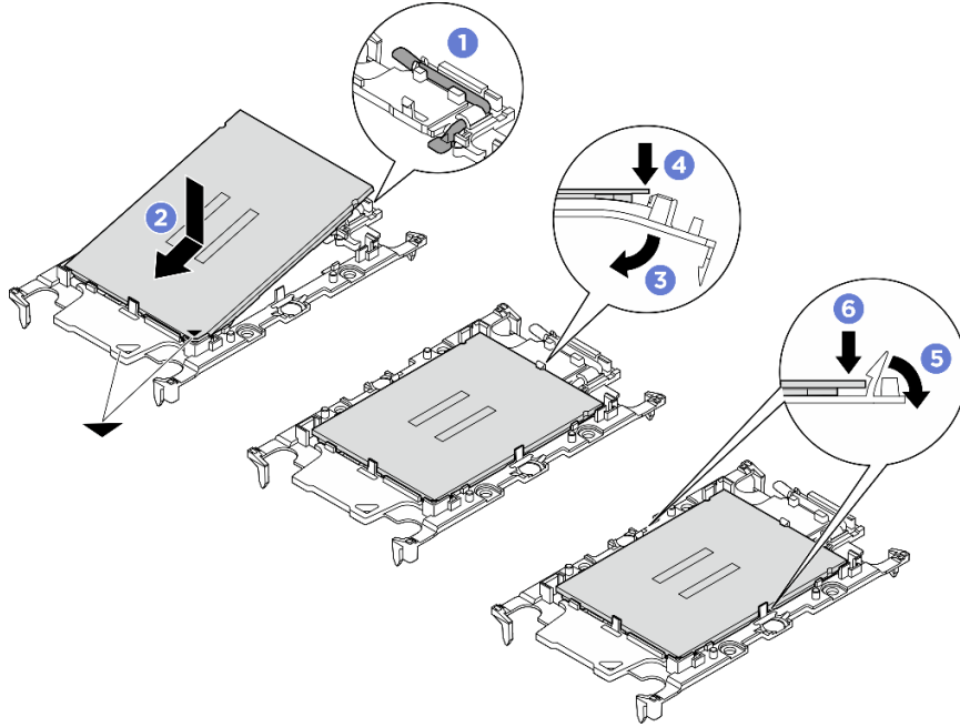
그림 105. 프로세서 캐리어 설치
