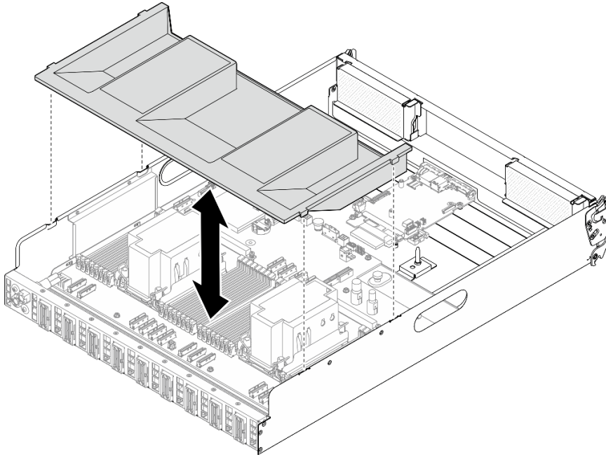
그림 95. 프로세서 공기 조절 장치 제거
