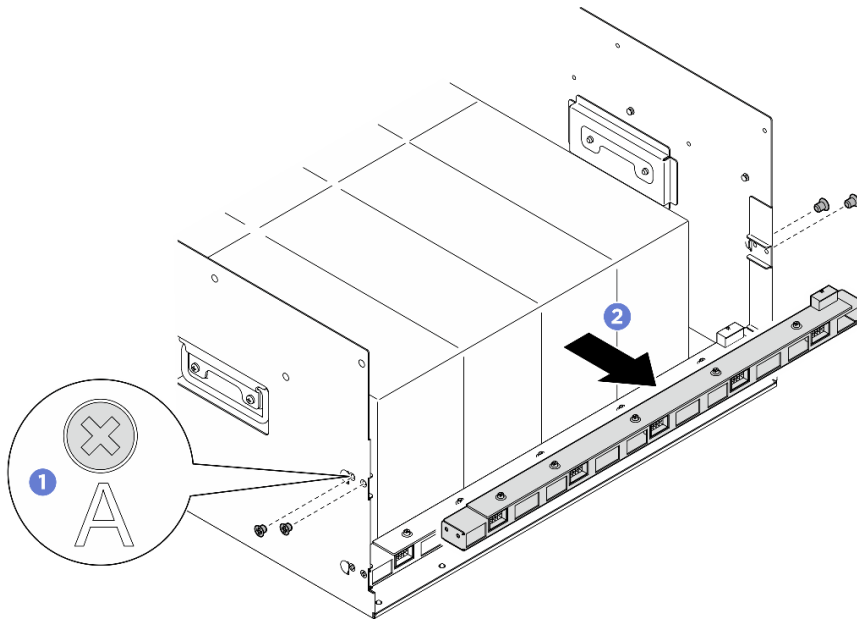
그림 56. 뒷면 팬 컨트롤 보드 어셈블리 제거
