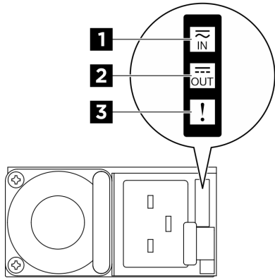
รูปภาพ 12. ไฟ LED แหล่งจ่ายไฟ CFFv4
