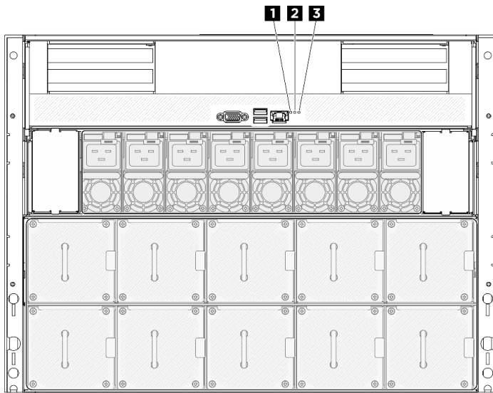
รูปภาพ 13. ไฟ LED ระบบที่มุมมองด้านหลัง
