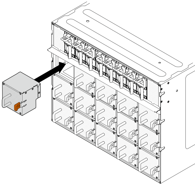
Figura 68. Installazione della ventola posteriore
