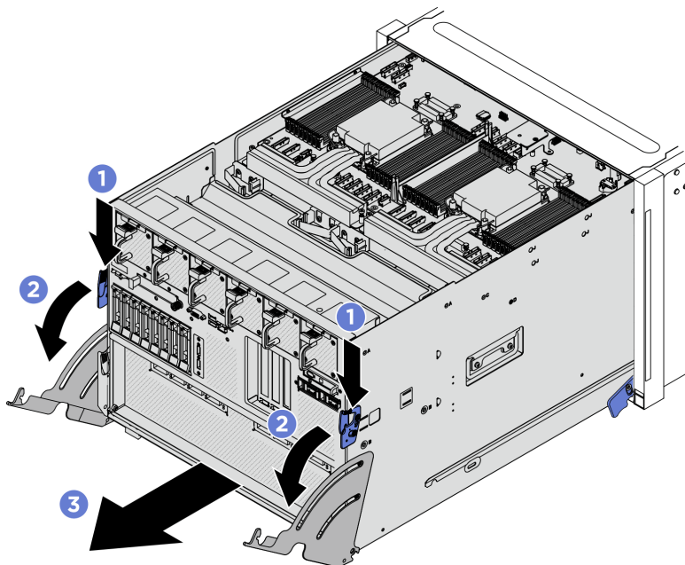
Figura 28. Trazione dello shuttle di sistema in posizione di arresto
