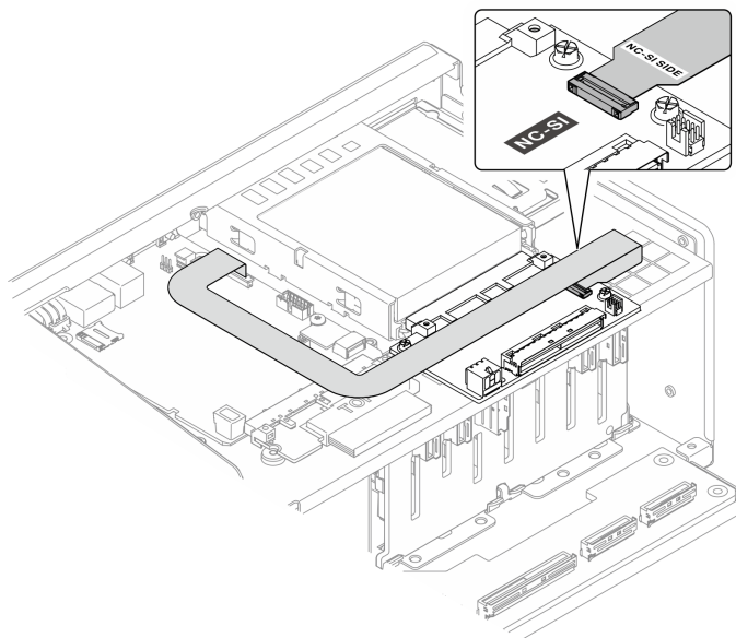
Figura 175. Collegamento del cavo FPC
