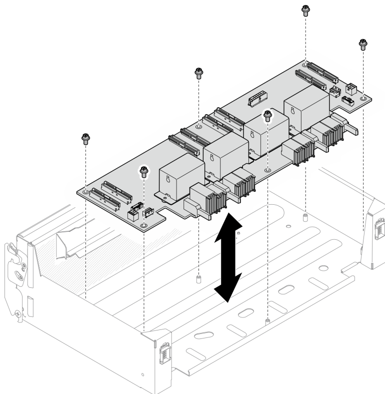
Figura 267. Installazione della scheda retimer
