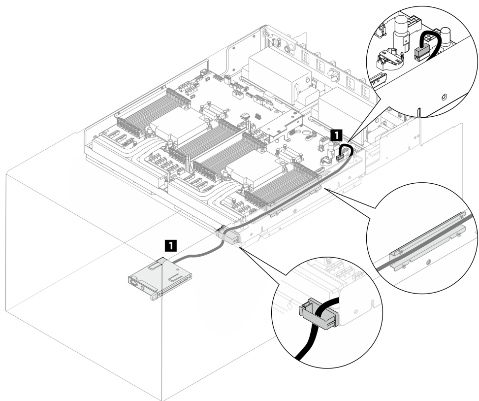
Figura 321. Instradamento del cavo del pannello di diagnostica integrato
