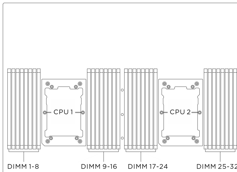
Figura 167. Layout dei moduli di memoria e dei processori
