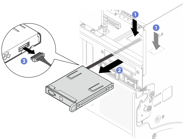
Figura 142. Rimozione del pannello di diagnostica integrato
