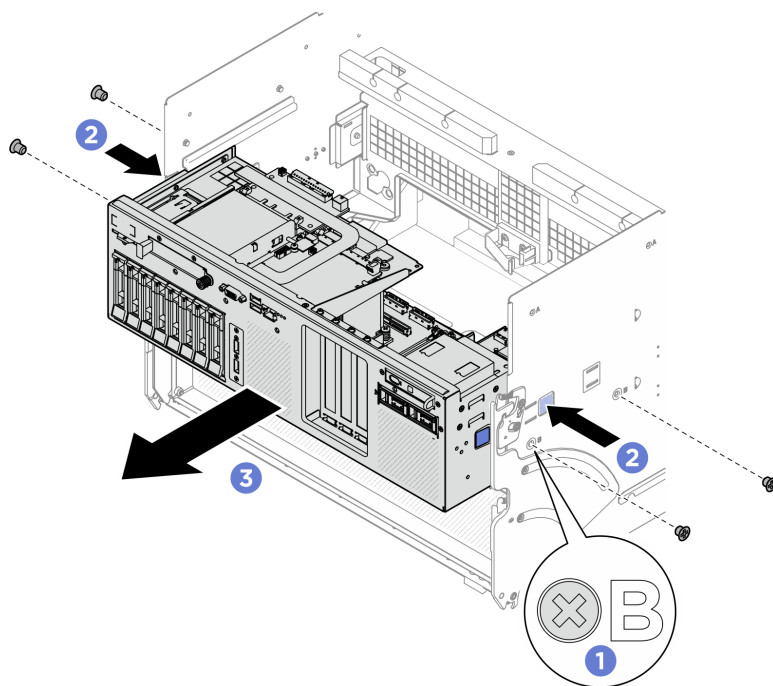
Figura 49. Trazione del telaio dell'unità NVMe e della scheda dello switch PCIe fino alla posizione di blocco
