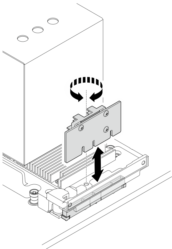
Figura 139. Installazione della scheda HMC
