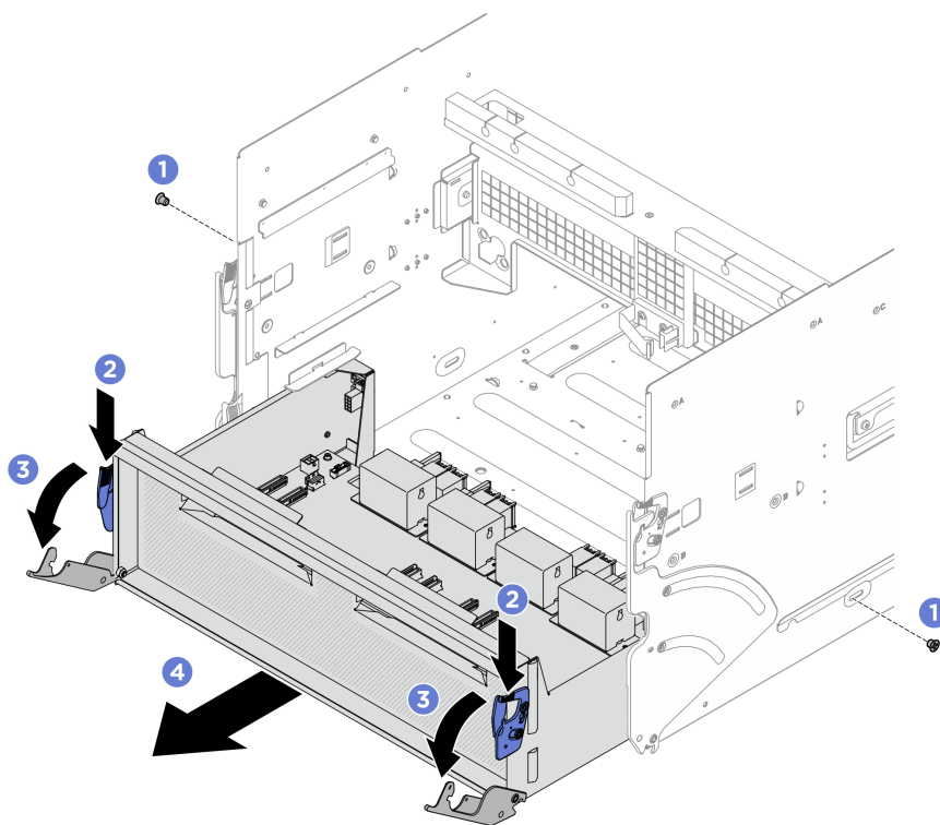
Figura 271. Rimozione dello shuttle della scheda retimer
