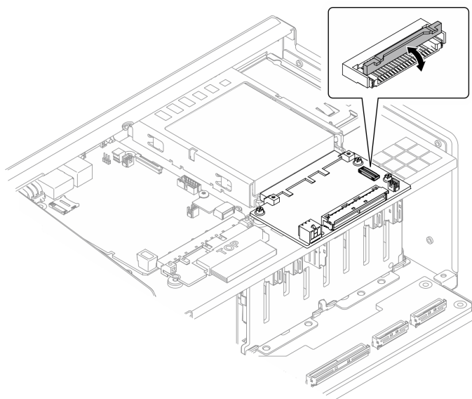
Figura 171. Sollevamento della linguetta del connettore
