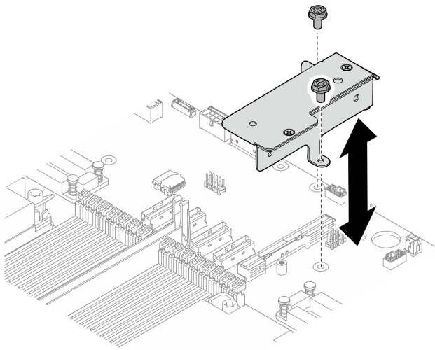
Figura 35. Installazione della guida per il cavo centrale
