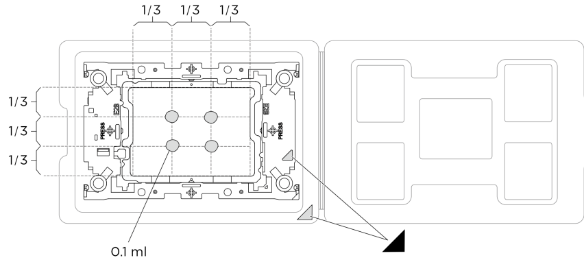
Figura 253. Applicazione del lubrificante termico con il processore nella confezione di spedizione
