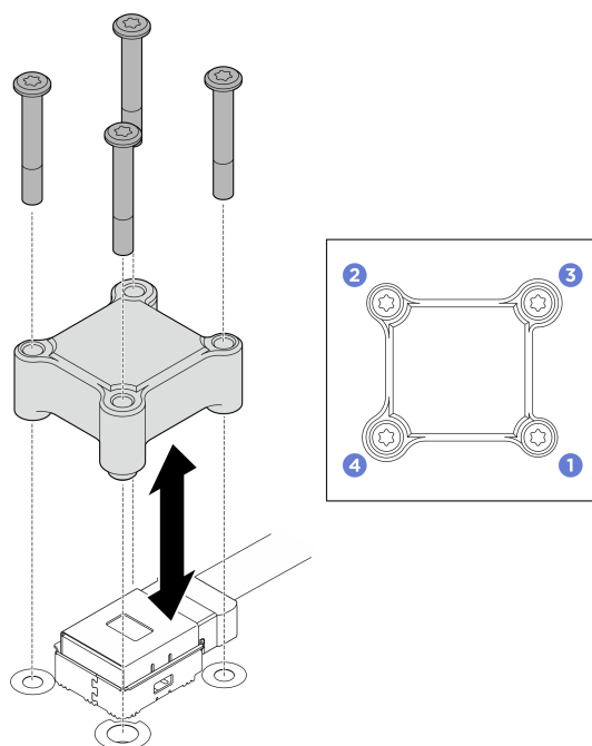
Figura 189. Rimozione del cappuccio del connettore
