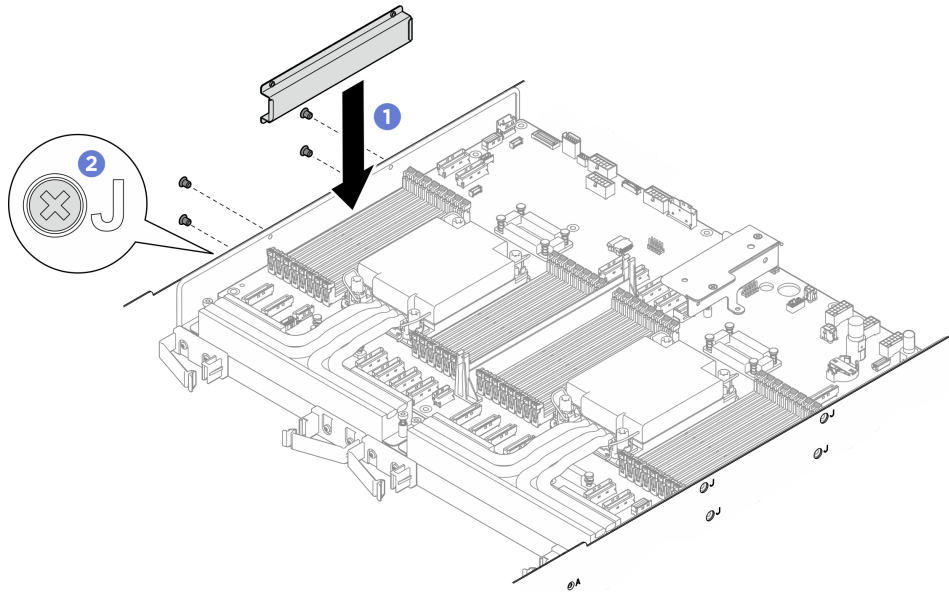
Figura 32. Installazione della guida per il cavo sinistra
