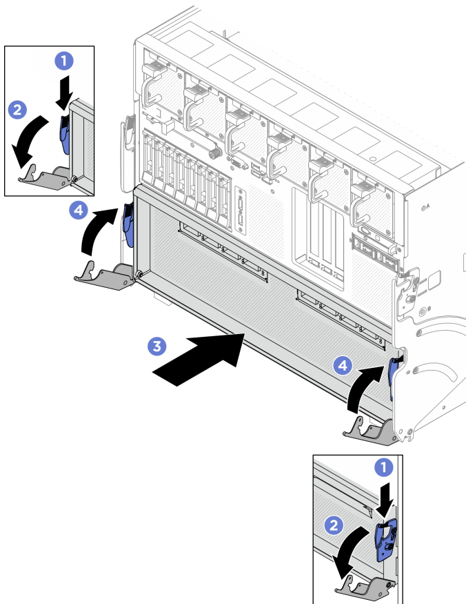
Figura 279. Aggancio dello shuttle della scheda retimer
