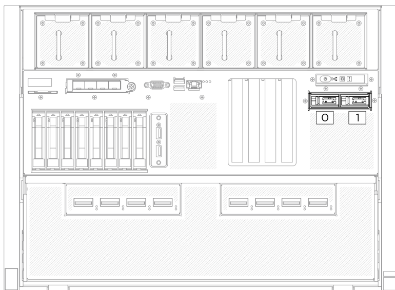
Figura 147. Numerazione dei vani delle unità M.2
