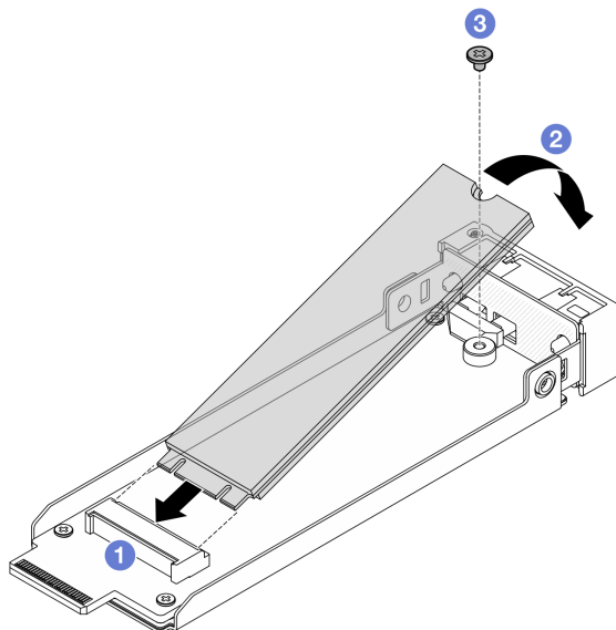
Figura 153. Installazione dell'unità M.2
