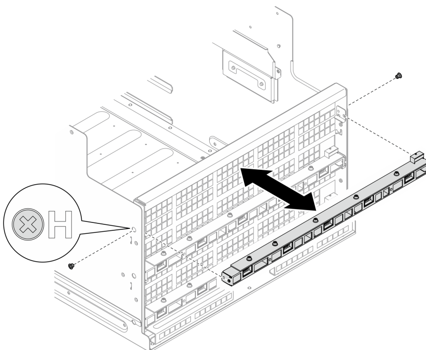
Figura 78. Installazione dell'assieme della scheda di controllo della ventola posteriore
