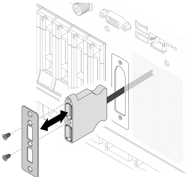
Figura 52. Rimozione della piastra dell'assieme USB
