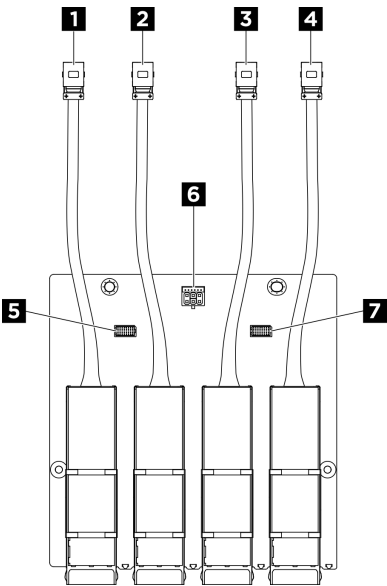
Figura 302. Cavi e connettori della scheda OSFP
