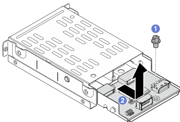
Figura 159. Rimozione del backplane M.2
