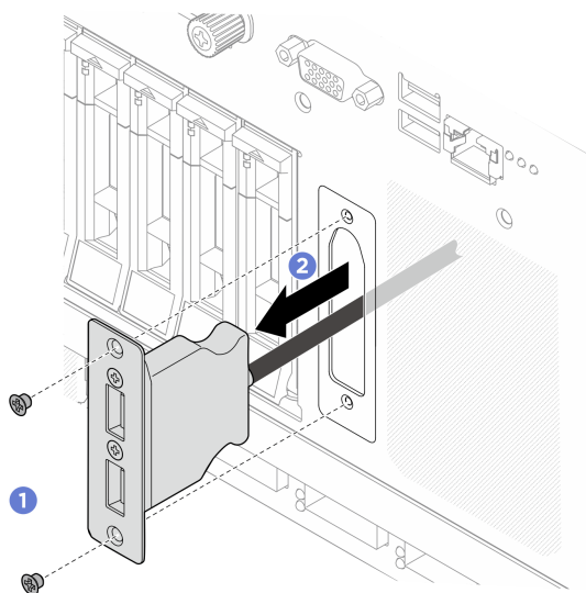
Figura 51. Rimozione dell'assieme USB
