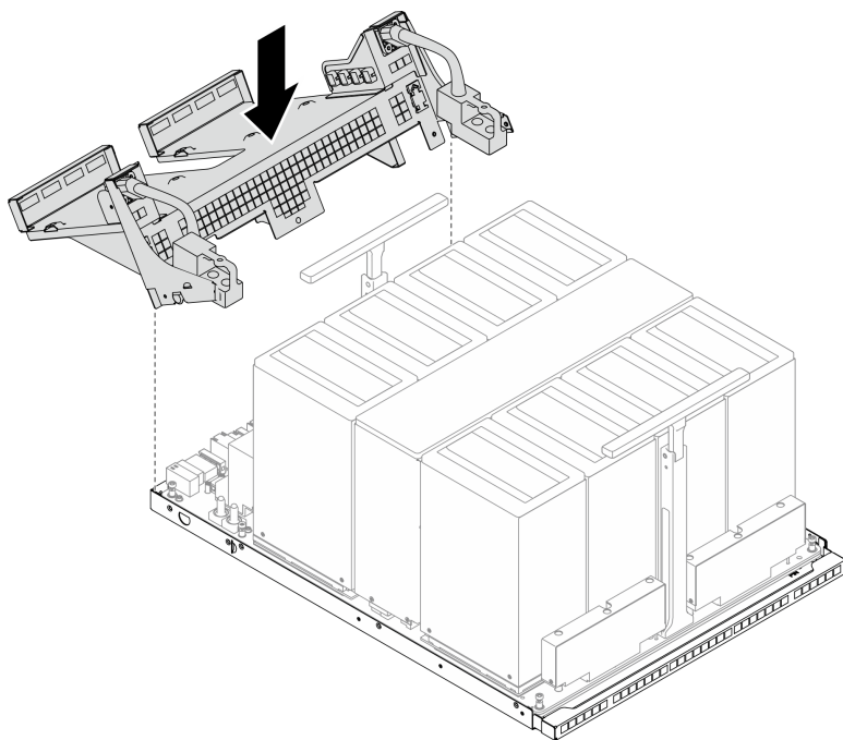
Figura 199. Installazione del vassoio di supporto OSFP
