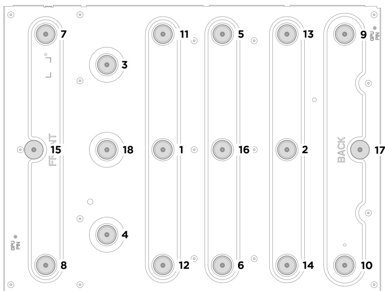
Figura 104. Sequenza di serraggio delle viti
