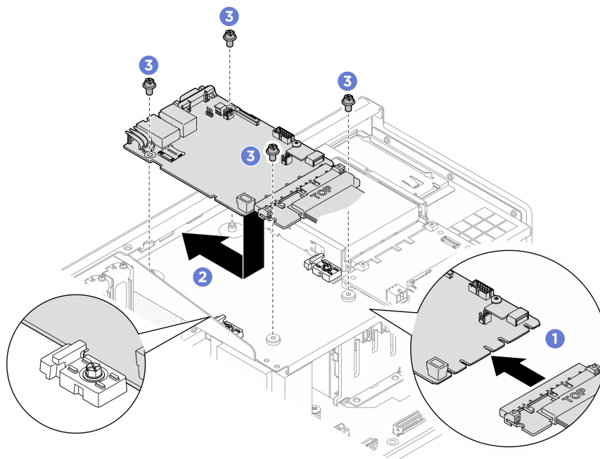
Figura 286. Installazione della scheda I/O di sistema
