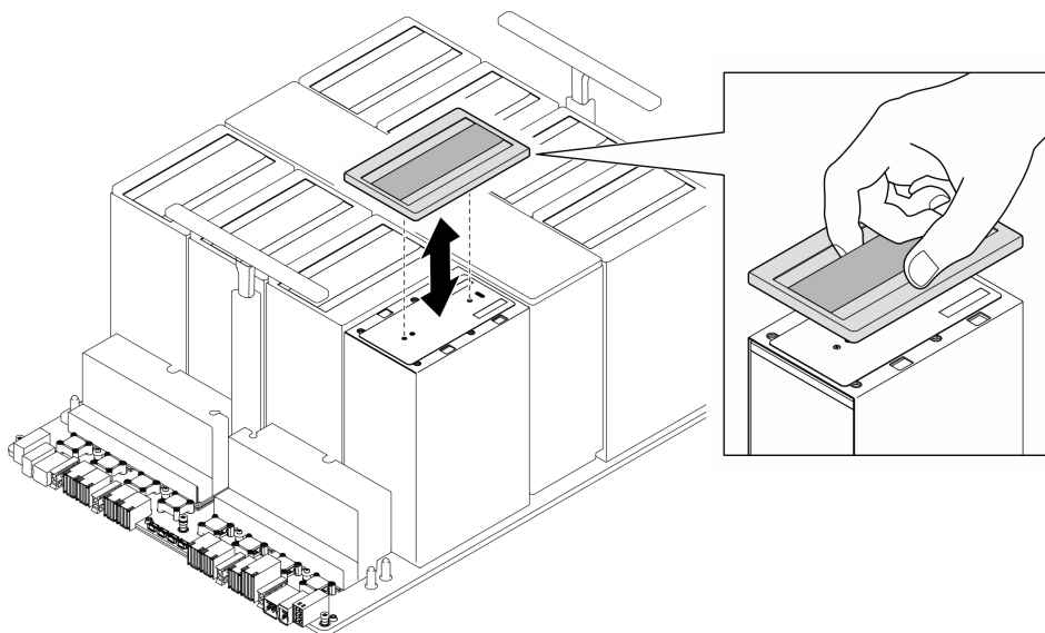
Figura 117. Installazione del coperchio in plastica
