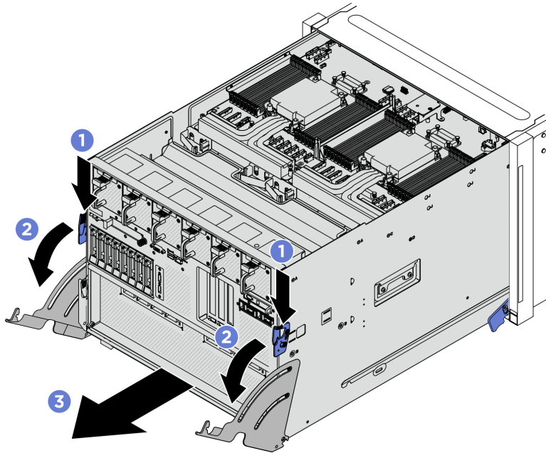
Figura 214. Trazione dello shuttle di sistema in posizione di arresto
