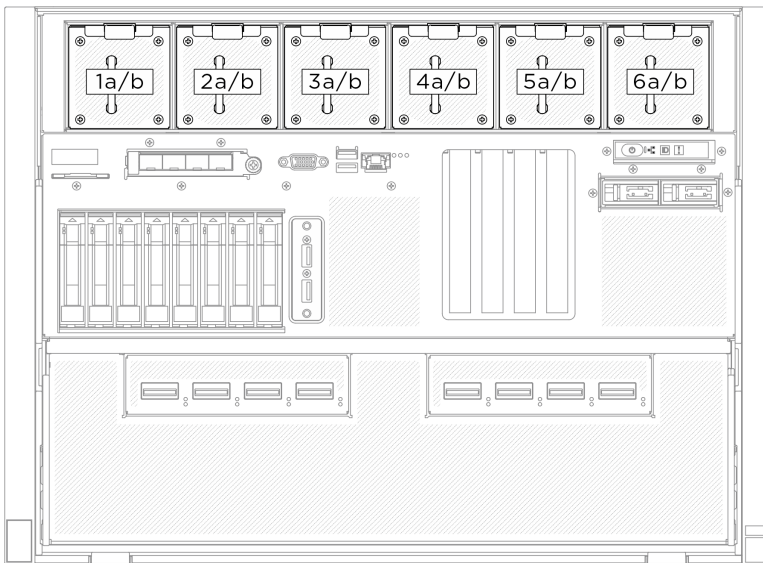
Figura 61. Numerazione delle ventole anteriori
