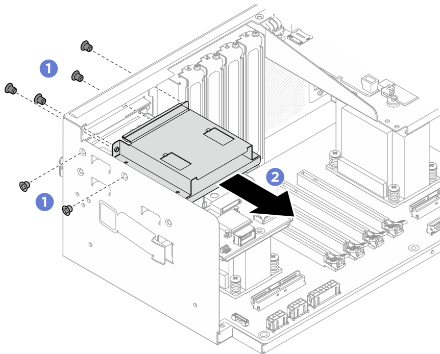
Figura 222. Rimozione del telaio del pannello di diagnostica integrato
