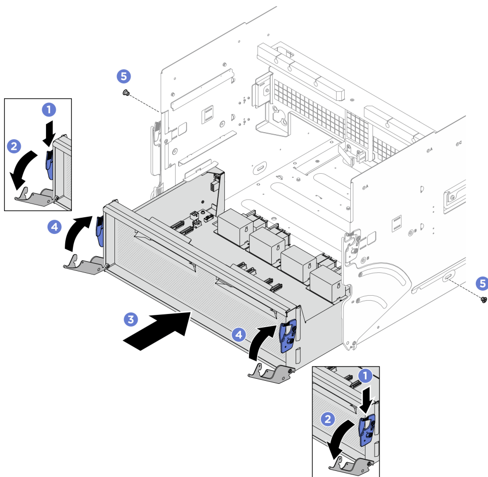
Figura 274. Installazione dello shuttle della scheda retimer
