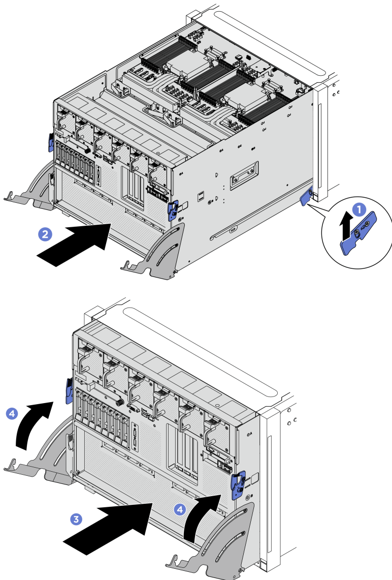
Figura 73. Installazione dello shuttle di sistema
