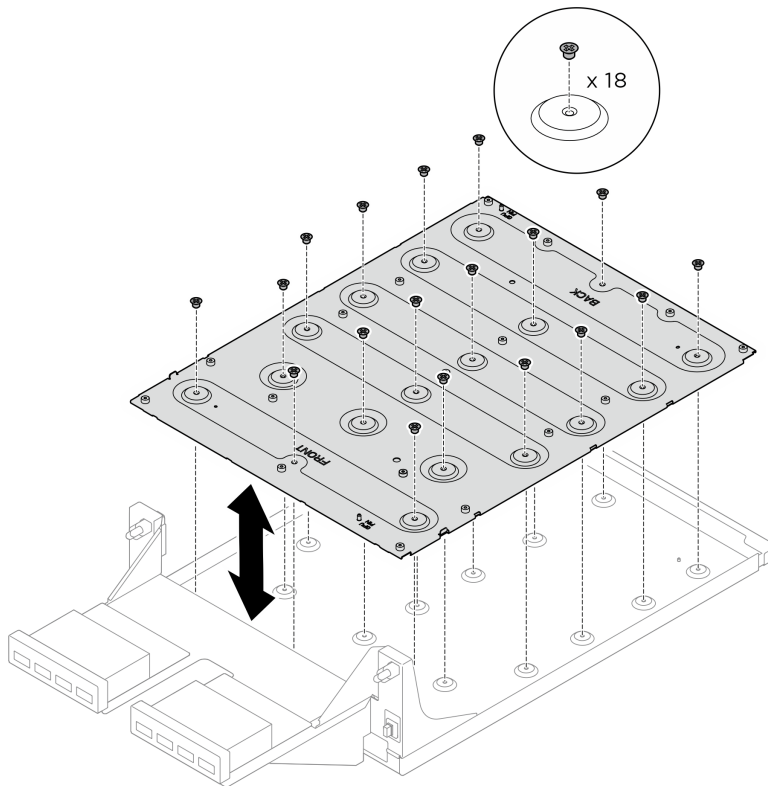
Figura 103. Installazione della piastra adattatore del complesso GPU
