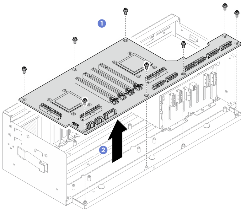
Figura 226. Rimozione della scheda dello switch PCIe
