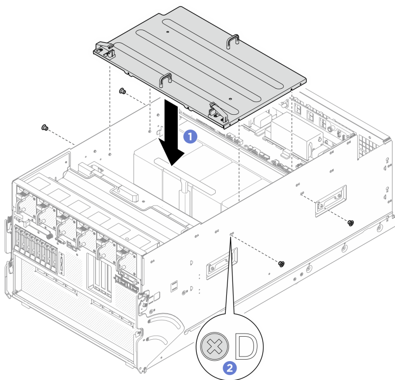
Figura 37. Installazione del telaio del fermacavo e dell'assieme del deflettore
