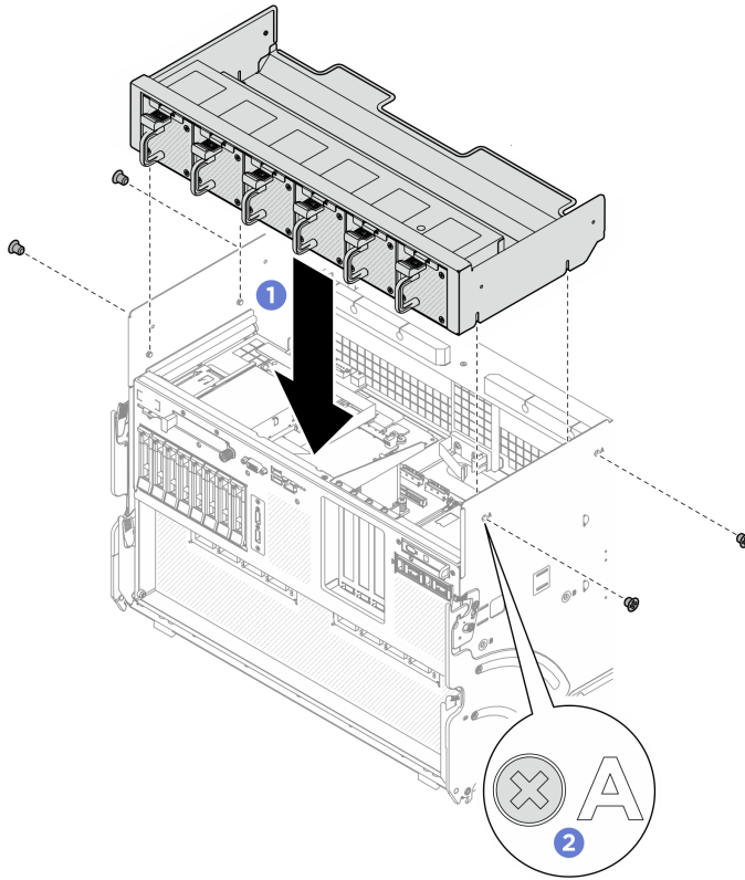
Figura 81. Installazione dell'alloggiamento della ventola anteriore
