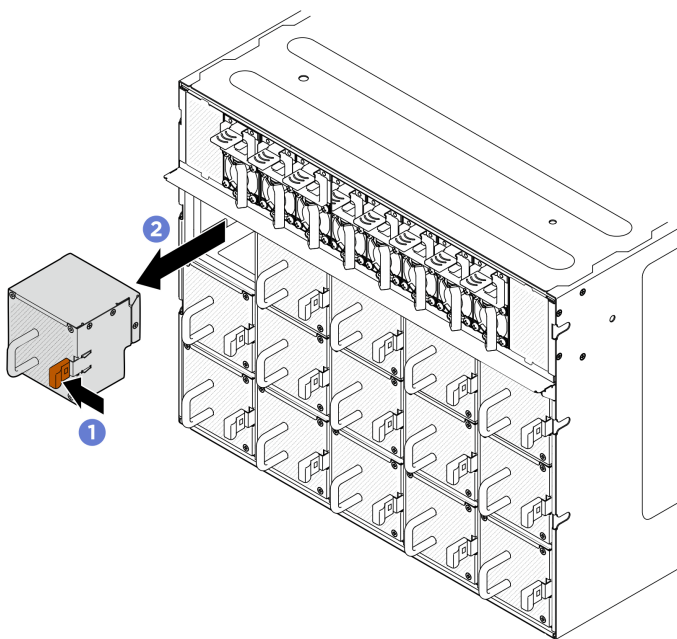
Figura 64. Rimozione della ventola posteriore
