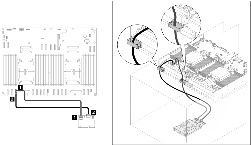
Figura 323. Instradamento dei cavi del backplane M.2
