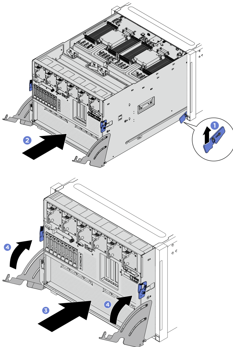
Figura 145. Installazione dello shuttle di sistema
