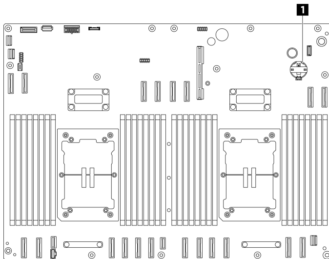
Figura 43. Posizione della batteria CMOS
