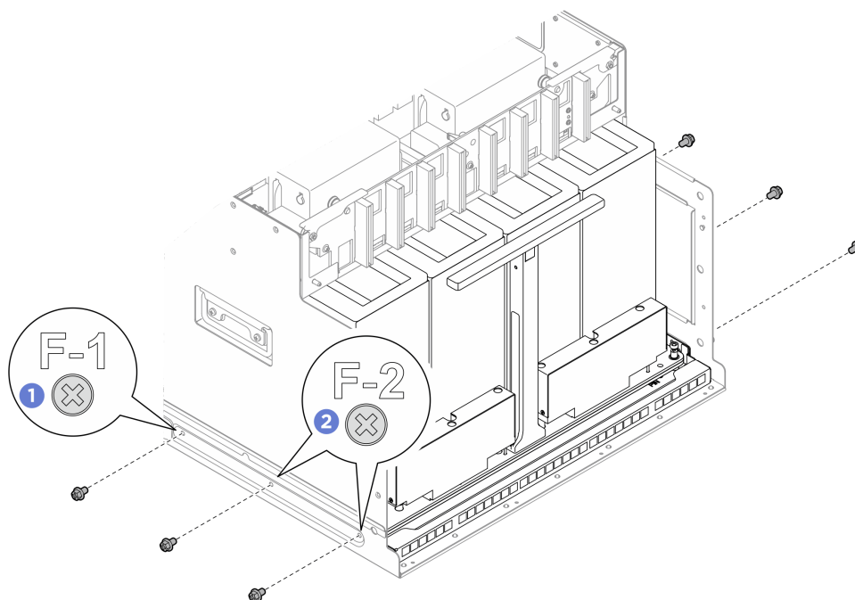
Figura 126. Installazione delle viti
