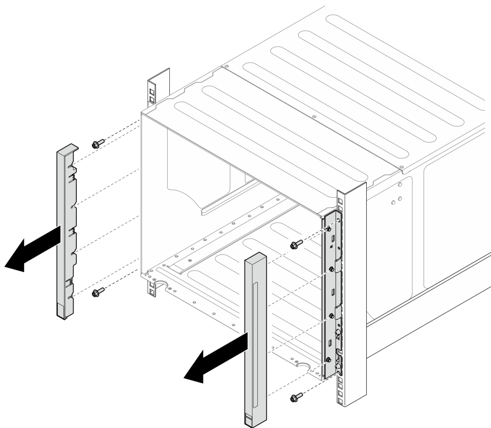
Figura 4. Rimozione del coperchio EIA
