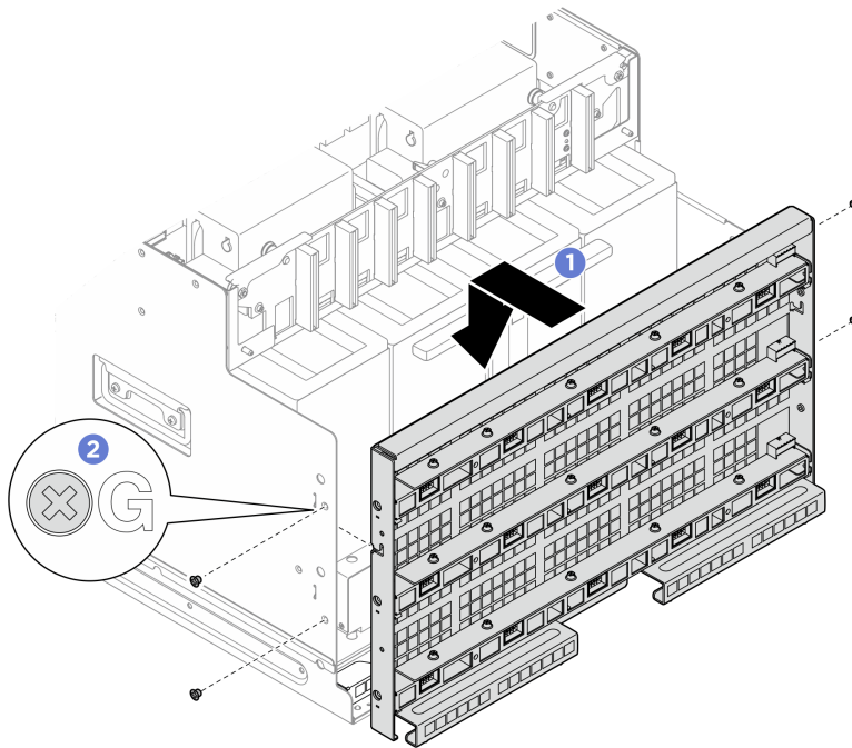
Figura 264. Installazione della paratia della ventola posteriore
