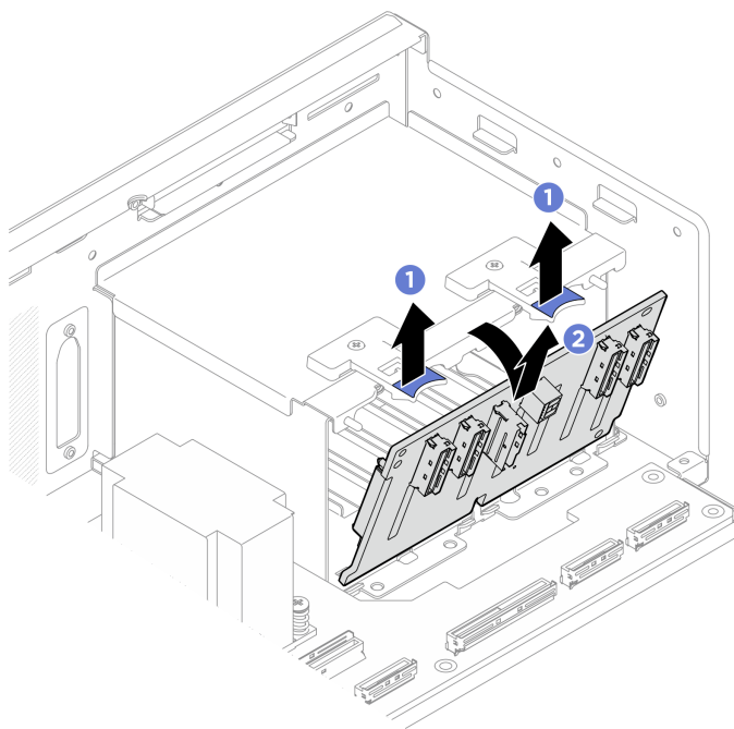
Figura 23. Rimozione del backplane dell'unità da 2,5 pollici
