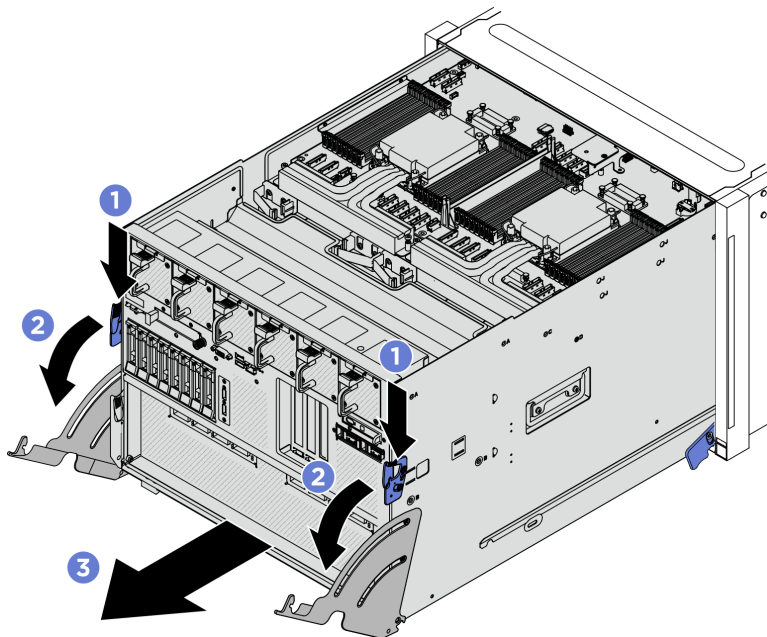
Figura 69. Trazione dello shuttle di sistema in posizione di arresto
