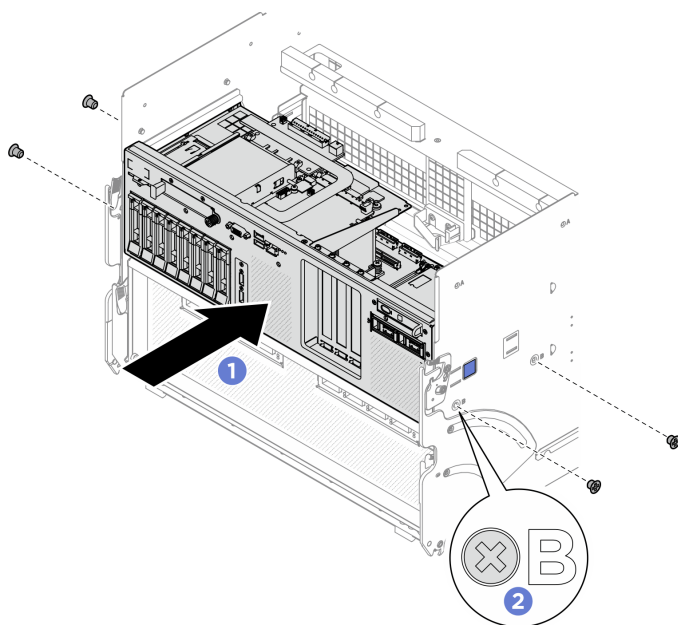
Figura 59. Installazione del telaio dell'unità NVMe e della scheda dello switch PCIe
