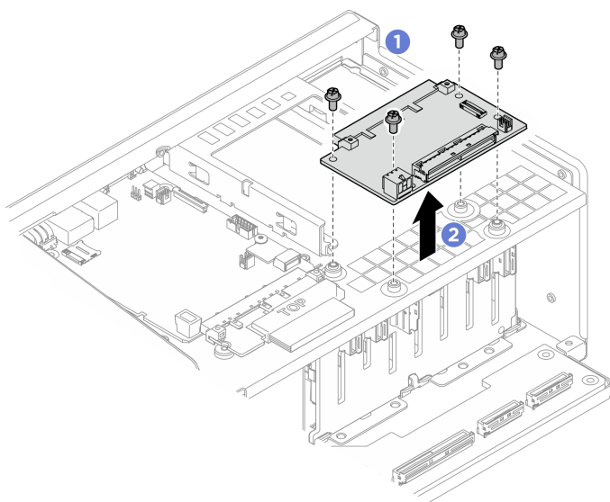
Figura 172. Rimozione della scheda interposer OCP
