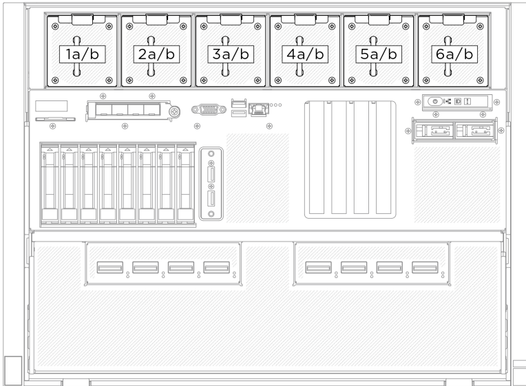
Figura 65. Numerazione delle ventole anteriori
