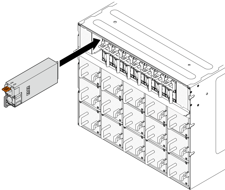
Figura 242. Installazione dell'unità di alimentazione
