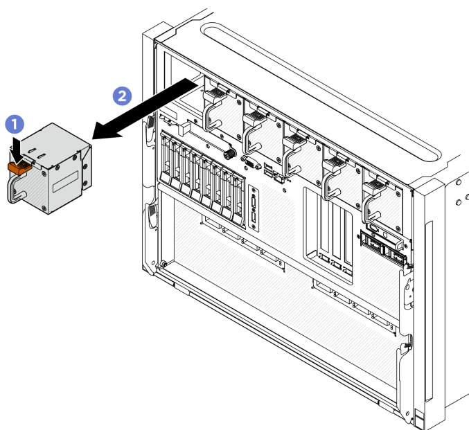
Figura 63. Rimozione della ventola anteriore
