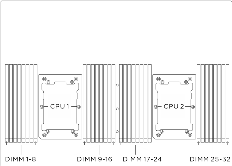
Figura 1. Layout dei moduli di memoria e dei processori
