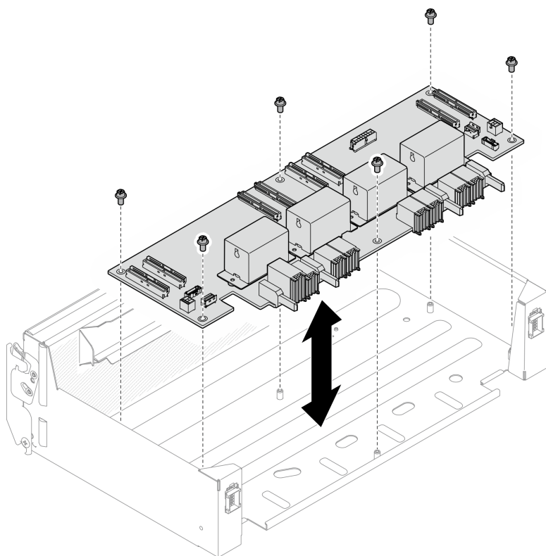
Figura 266. Rimozione della scheda retimer
