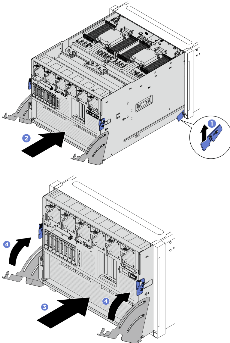
Figura 269. Installazione dello shuttle di sistema
