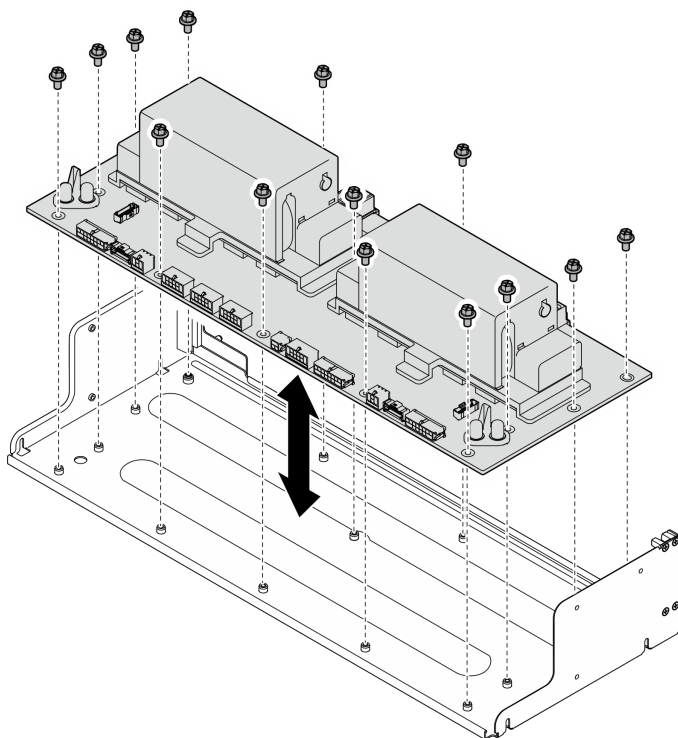
Figura 237. Rimozione della scheda di distribuzione dell'alimentazione
