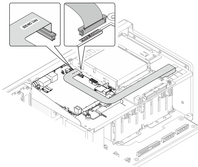
Figura 288. Collegamento del cavo FPC
