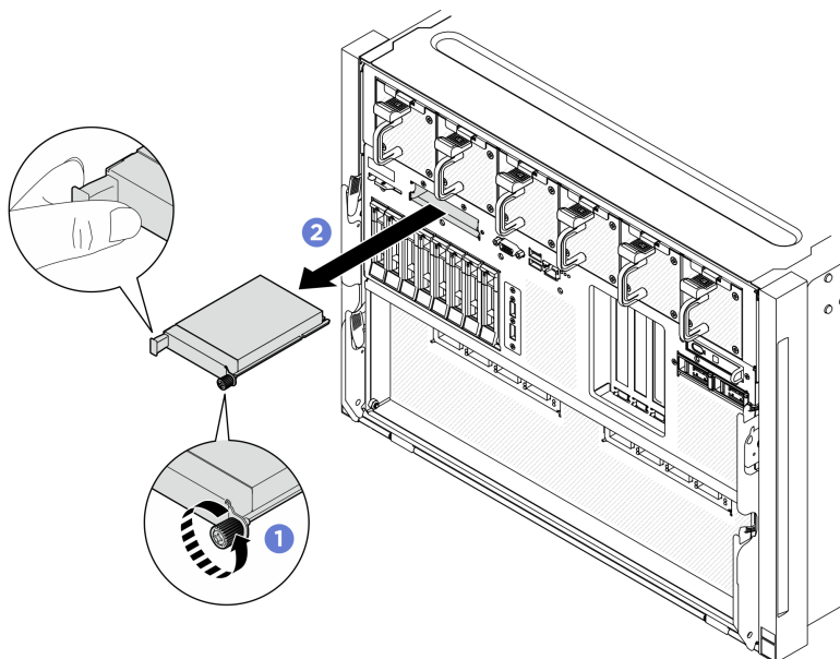
Figura 182. Rimozione del modulo OCP
