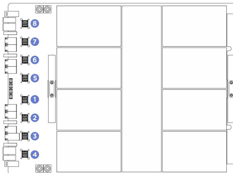
Figura 188. Sequenza di rimozione dei cavi UltraPass
