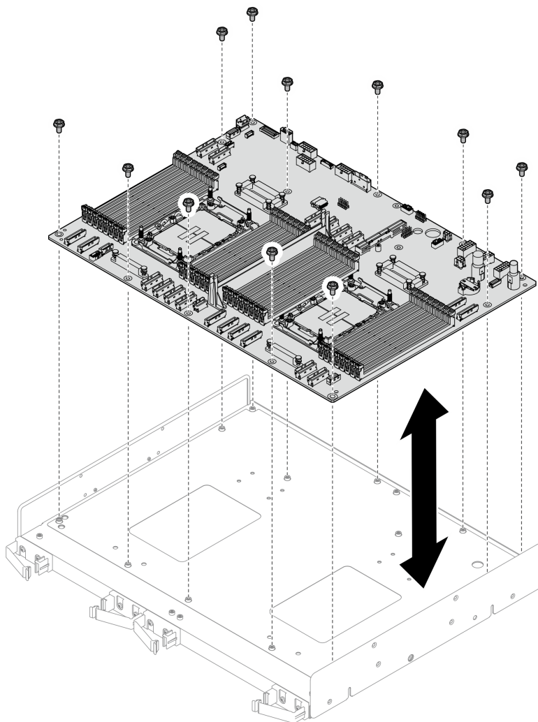
Figura 281. Installazione della scheda di sistema
