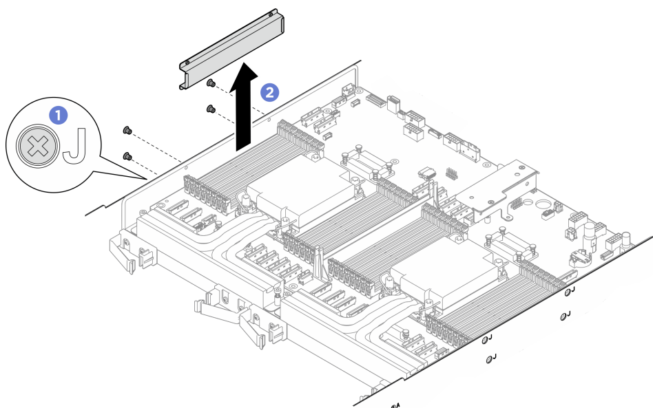
Figura 29. Rimozione della guida per il cavo sinistra
