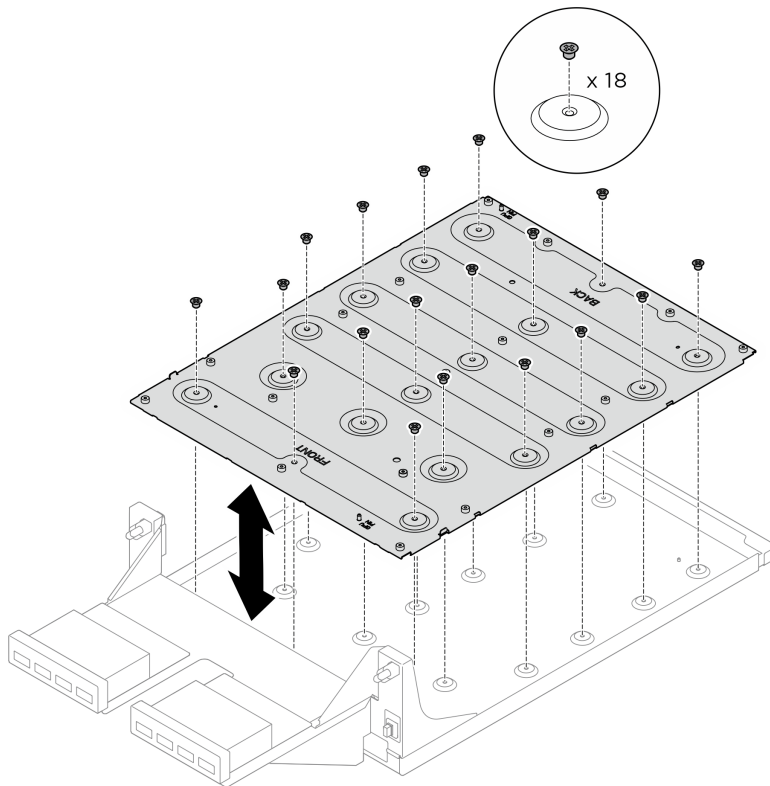
Figura 132. Installazione della piastra adattatore del complesso GPU
