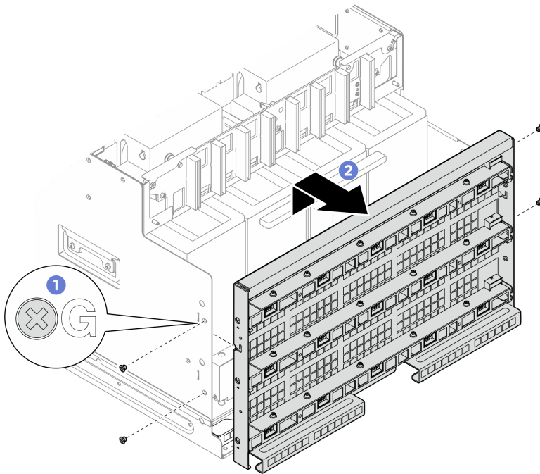
Figura 261. Sganciamento della paratia della ventola posteriore
