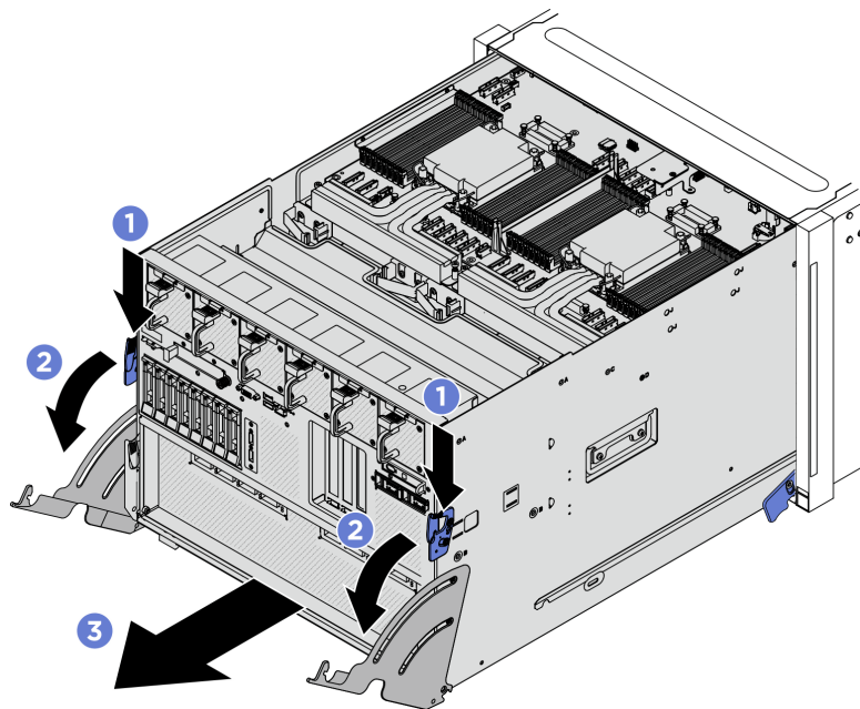
Figura 164. Trazione dello shuttle di sistema in posizione di arresto
