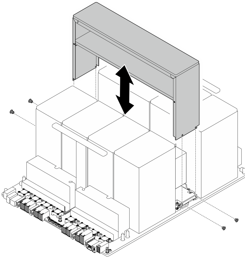
Figura 95. Rimozione del coperchio del dissipatore di calore NVSwitch
