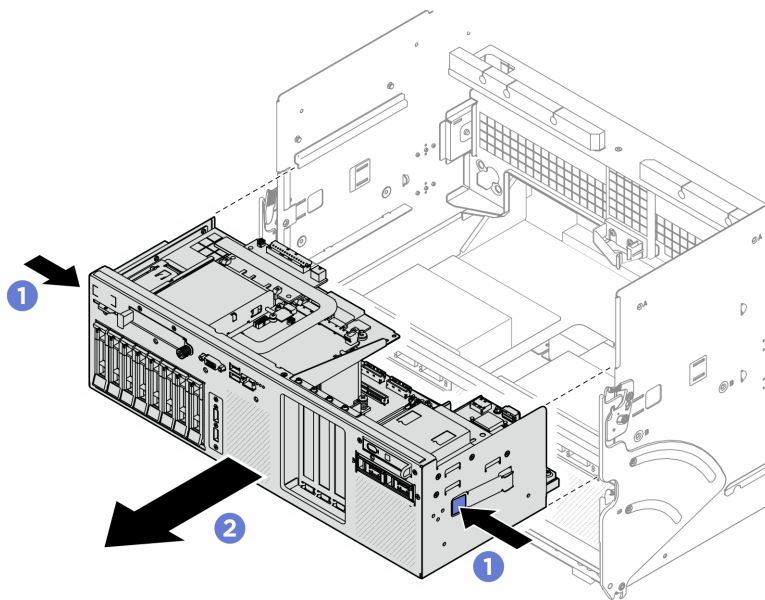
Figura 54. Rimozione del telaio dell'unità NVMe e della scheda dello switch PCIe
