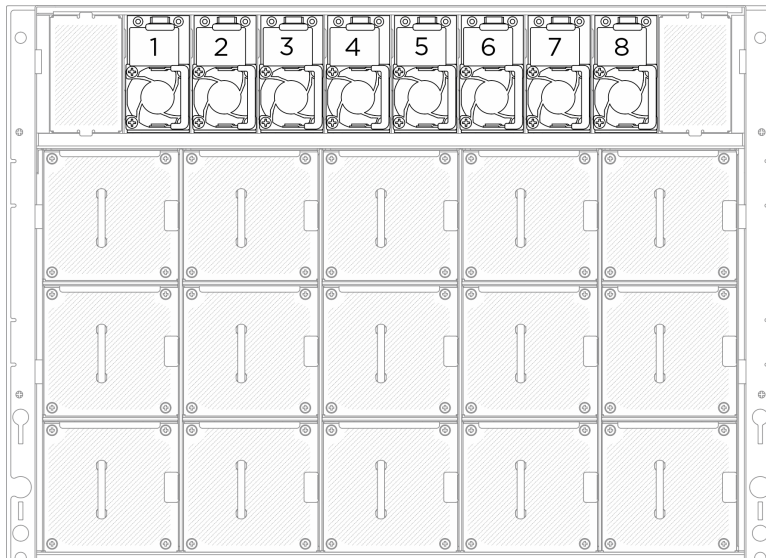
Figura 241. Numerazione del vano dell'alimentatore
