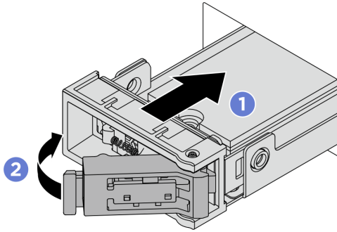
Figura 156. Installazione di un assieme dell'unità M.2
