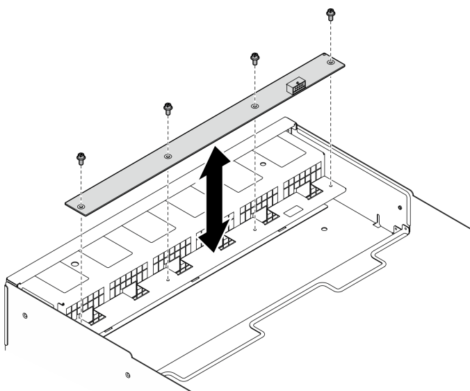
Figura 71. Installazione della scheda di controllo della ventola anteriore
