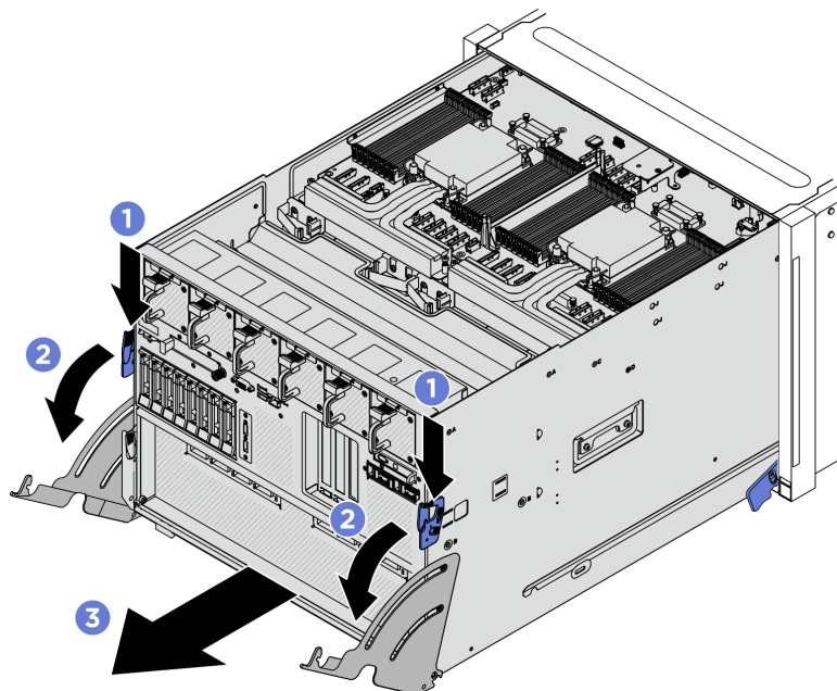
Figura 221. Trazione dello shuttle di sistema in posizione di arresto
