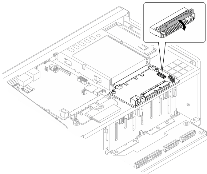
Figura 176. Abbassamento della linguetta del connettore
