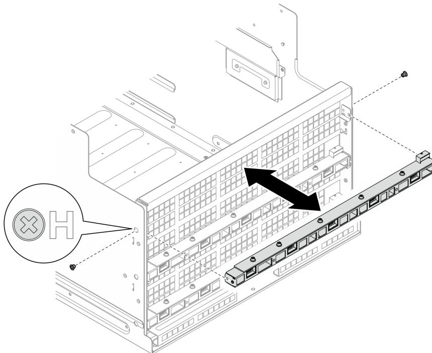
Figura 74. Rimozione dell'assieme della scheda di controllo della ventola posteriore
