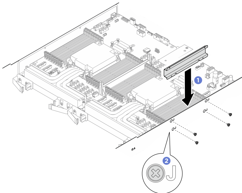
Figura 33. Installazione della guida per il cavo destra
