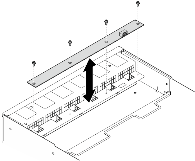
Figura 70. Rimozione della scheda di controllo della ventola anteriore
