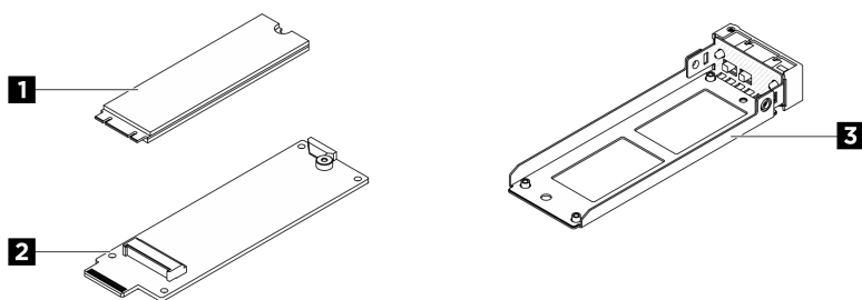
Figura 146. Parti di un assieme dell'unità M.2 hot-swap
