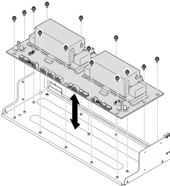
Figura 238. Installazione della scheda di distribuzione dell'alimentazione
