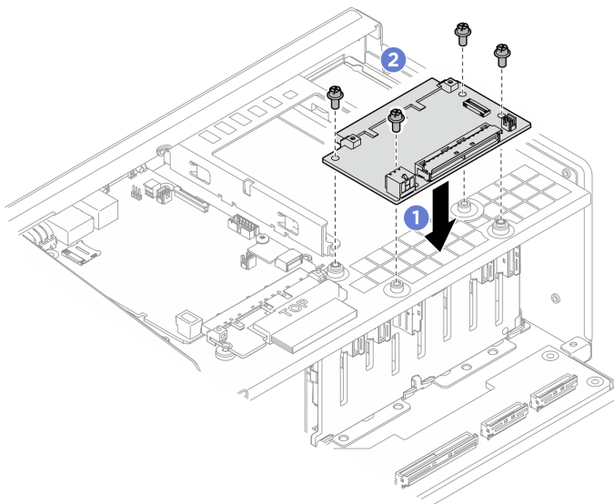
Figura 173. Installazione della scheda interposer OCP
