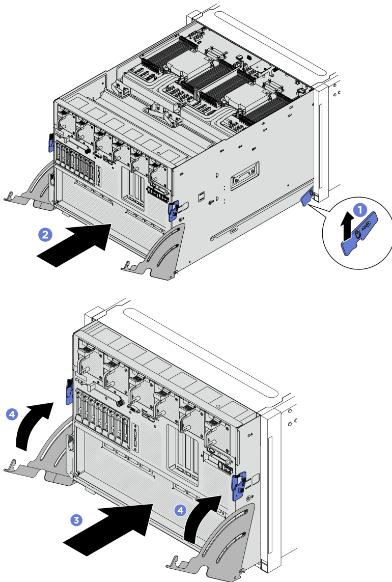
Figura 291. Installazione dello shuttle di sistema
