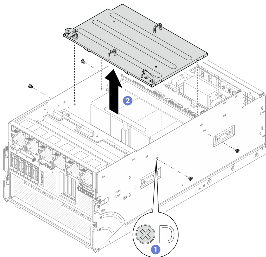
Figura 36. Rimozione del telaio del fermacavo e dell'assieme del deflettore
