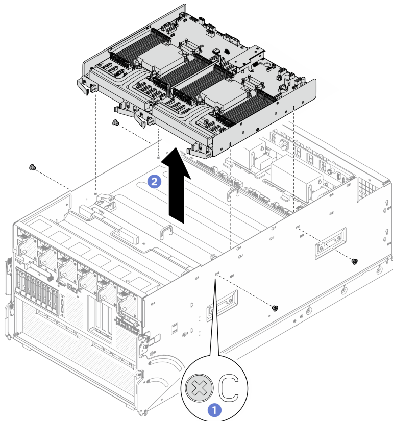
Figura 39. Rimozione del vassoio di elaborazione
