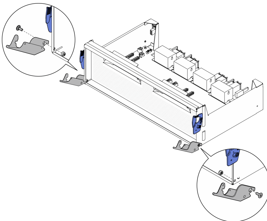
Figura 278. Installazione delle leve di rilascio della scheda retimer
