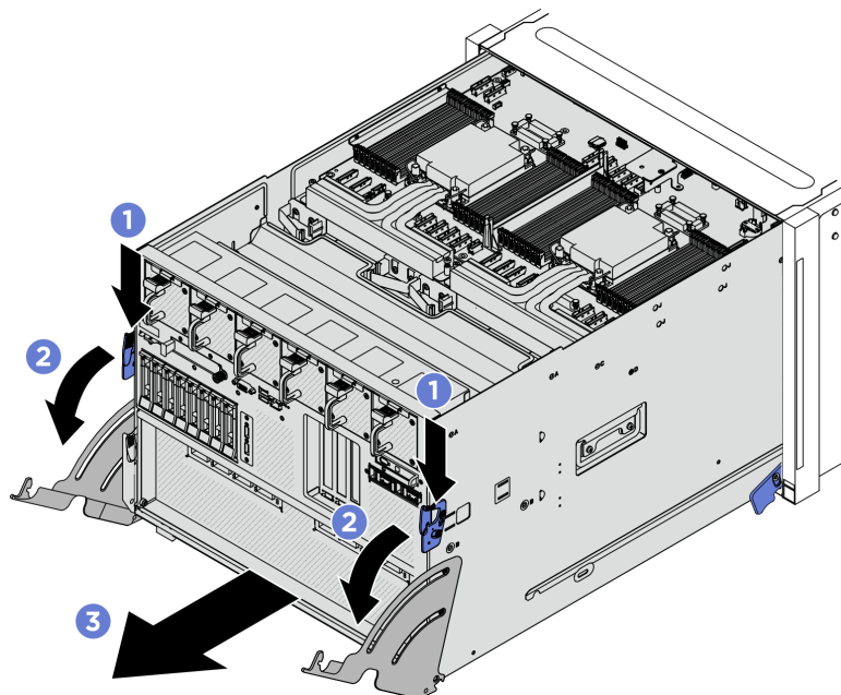
Figura 270. Trazione dello shuttle di sistema in posizione di arresto
