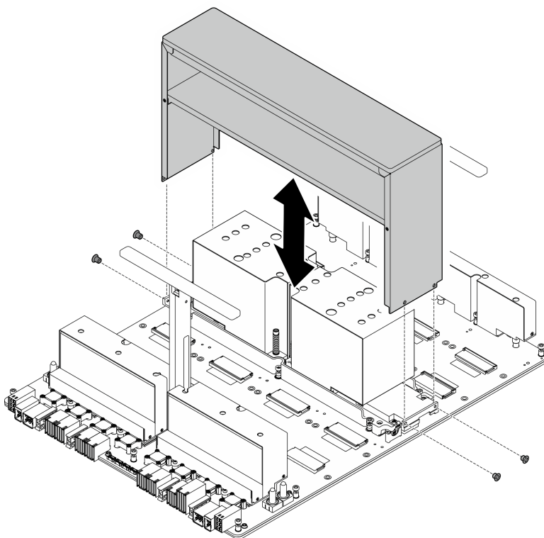
Figura 87. Rimozione del coperchio del dissipatore di calore NVSwitch
