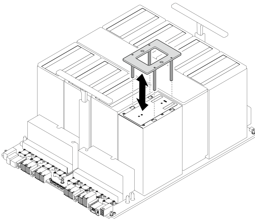
Figura 109. Installazione della dima
