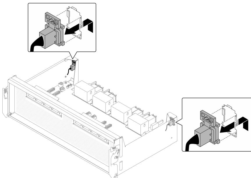
Figura 272. Rimozione del cavo laterale della scheda OSFP
