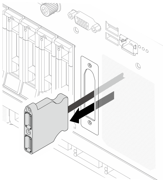
Figura 56. Installazione dell'assieme USB
