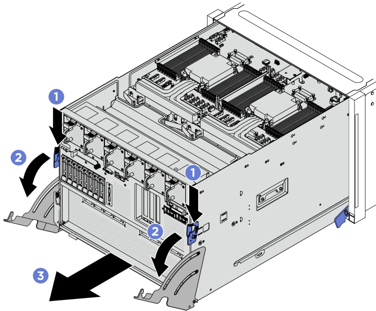
Figura 42. Trazione dello shuttle di sistema in posizione di arresto
