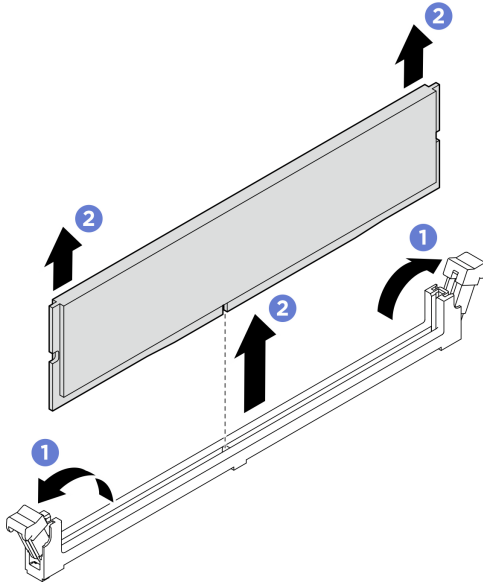
Figura 166. Rimozione del modulo di memoria
