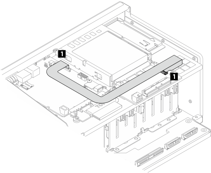
Figura 326. Instradamento del cavo dell'interfaccia NCSI (Network Controller Sideband Interface)
