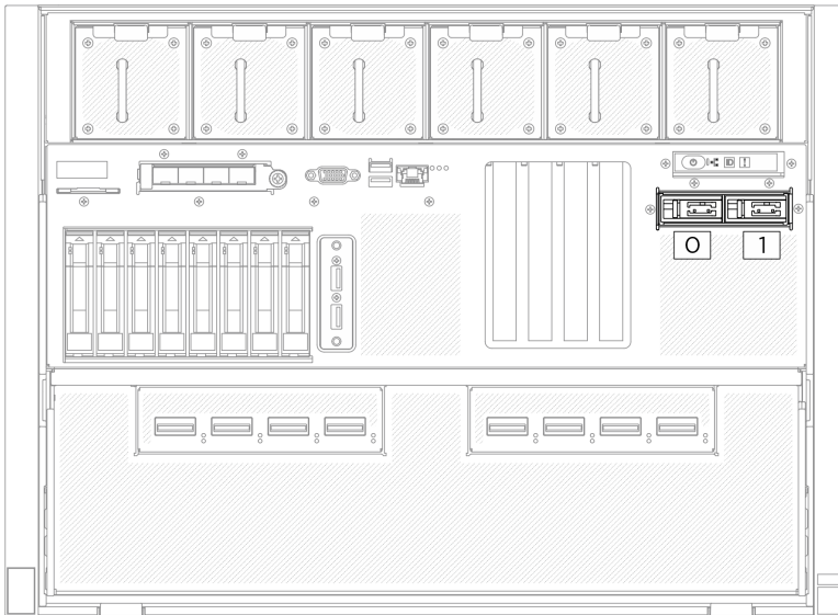
Figura 154. Numerazione dei vani delle unità M.2
