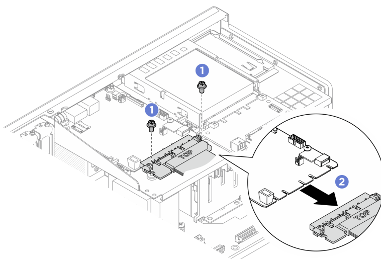
Figura 50. Rimozione del cavo della scheda I/O di sistema
