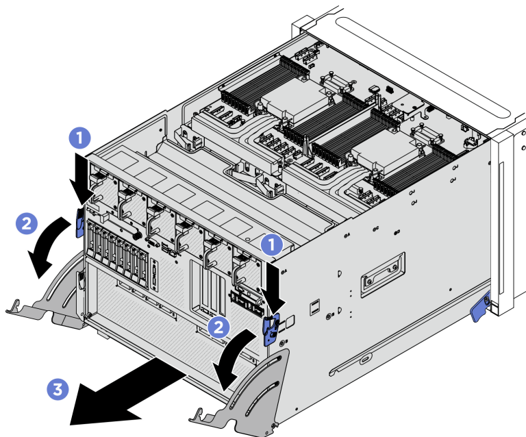
Figura 170. Trazione dello shuttle di sistema in posizione di arresto
