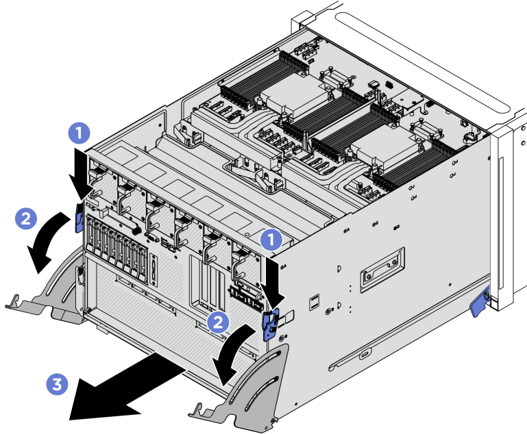
Figura 21. Trazione dello shuttle di sistema in posizione di arresto
