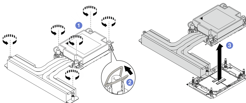
Figura 247. Rimozione del PHM
