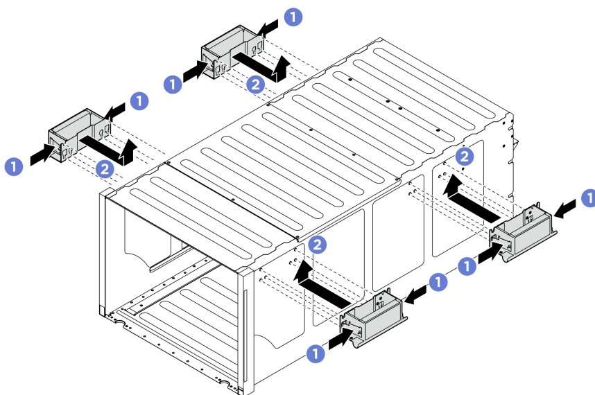
Figura 10. Fissaggio delle quattro maniglie
