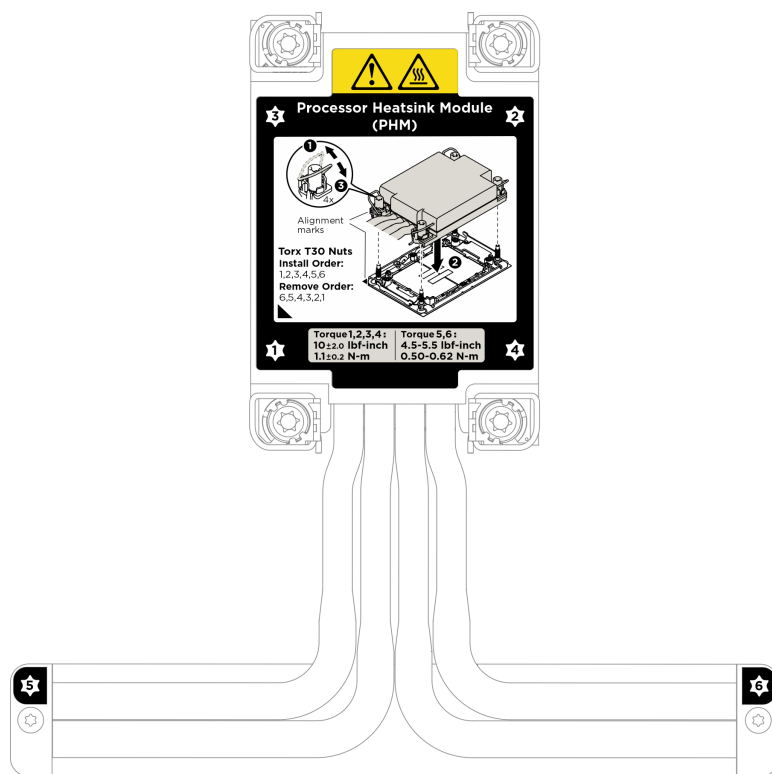
Figura 257. Etichetta del dissipatore di calore
