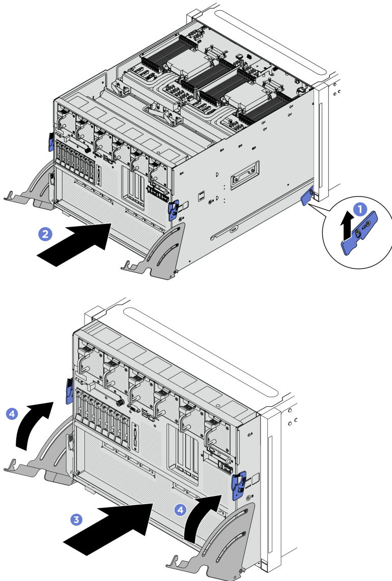
Figura 229. Installazione dello shuttle di sistema
