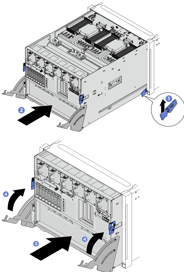
Figura 82. Installazione dello shuttle di sistema
