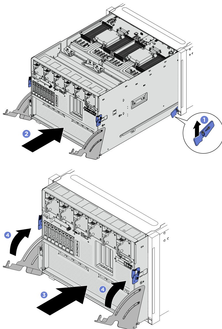
Figura 169. Installazione dello shuttle di sistema
