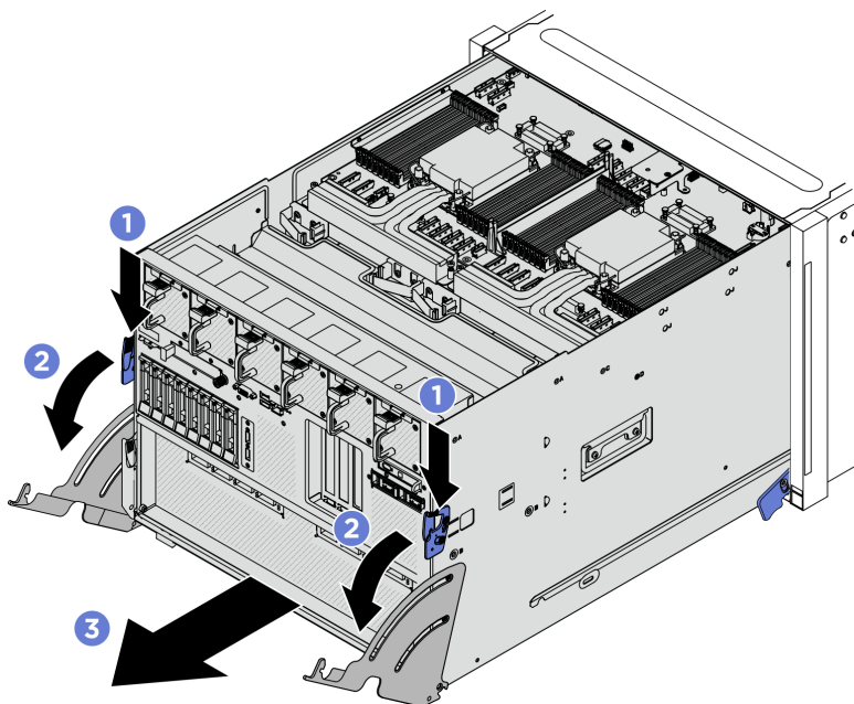
Figura 79. Trazione dello shuttle di sistema in posizione di arresto
