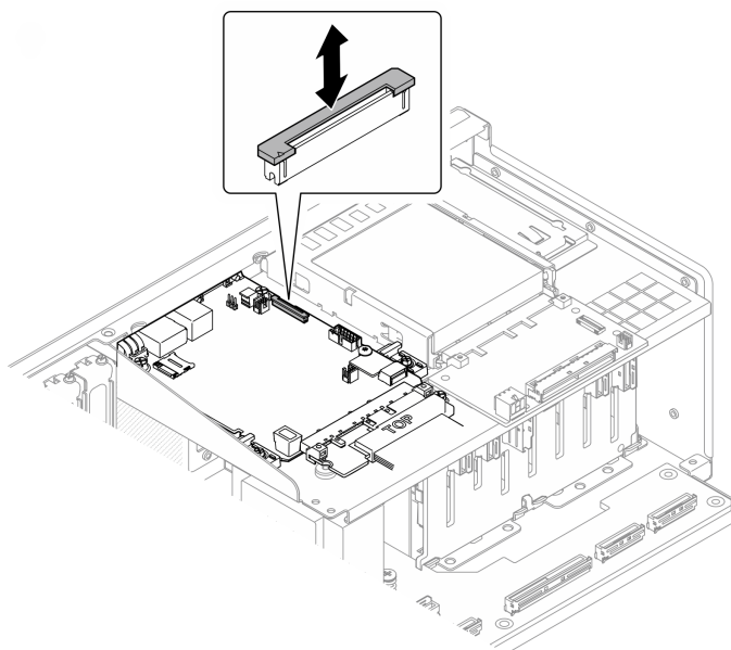
Figura 287. Sollevamento del fermo del connettore
