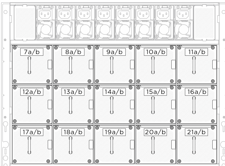
Figura 62. Numerazione delle ventole posteriori
