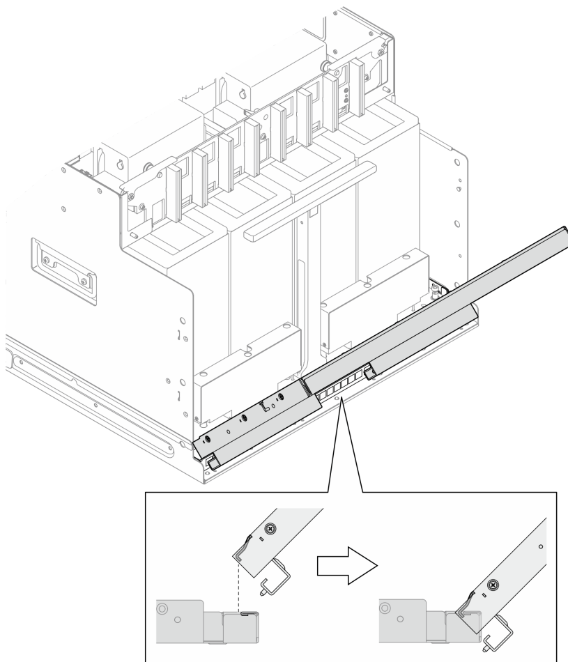
Figura 263. Aggancio della paratia della ventola posteriore alla staffa dello shuttle della GPU
