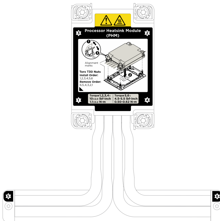
Figura 248. Etichetta del dissipatore di calore
