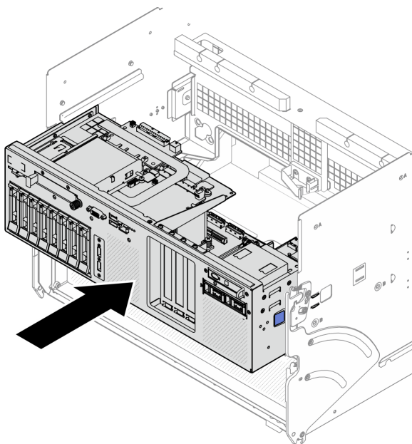
Figura 55. Inserimento del telaio dell'unità NVMe e della scheda dello switch PCIe in posizione di arresto
