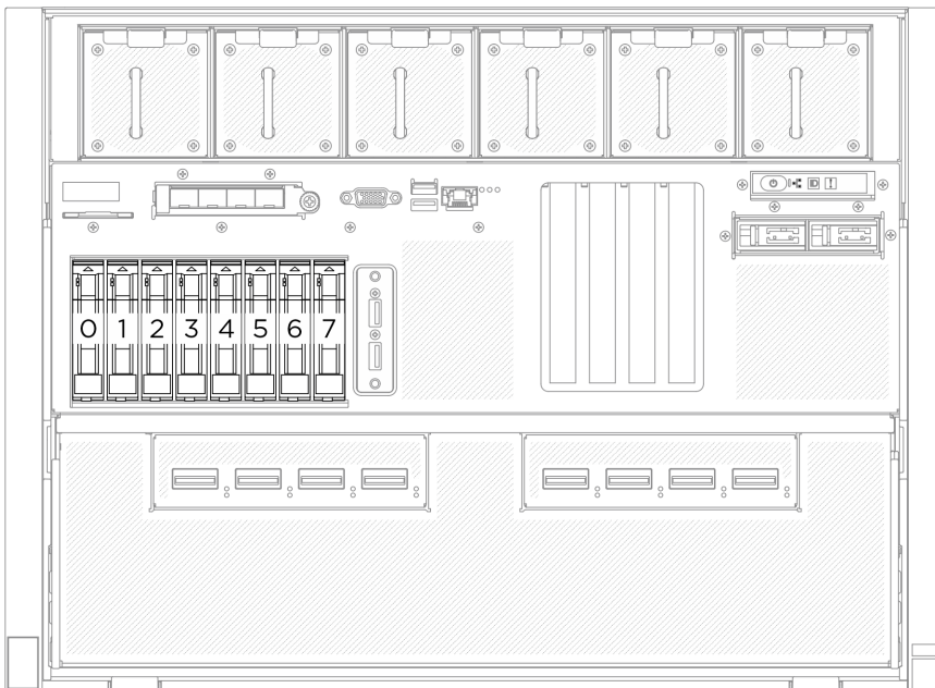
Figura 17. Numerazione del vano dell'unità da 2,5 pollici
