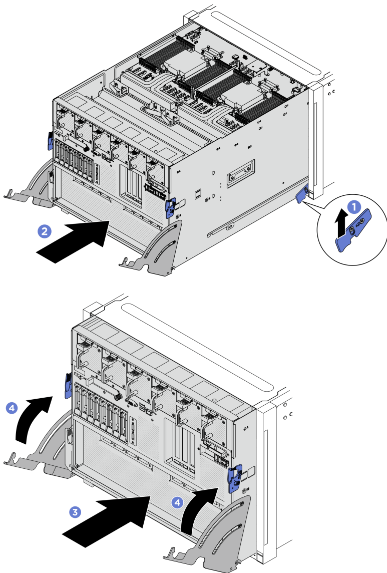
Figura 34. Installazione dello shuttle di sistema
