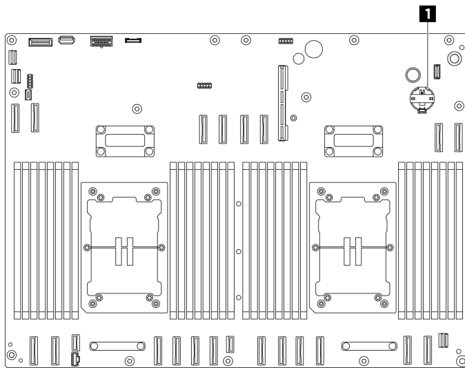
Figura 45. Posizione della batteria CMOS
