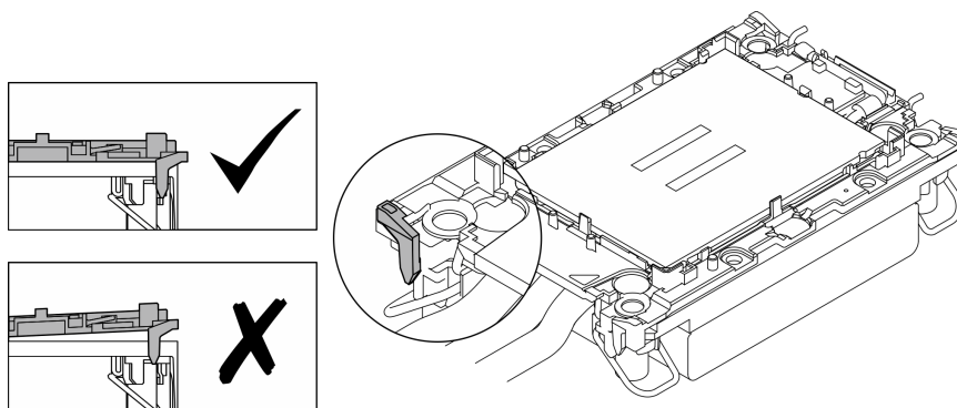
Figura 255. Controllo visivo dei fermi della piastra
