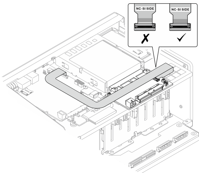
Figura 177. Ispezione dell'installazione del cavo FPC
