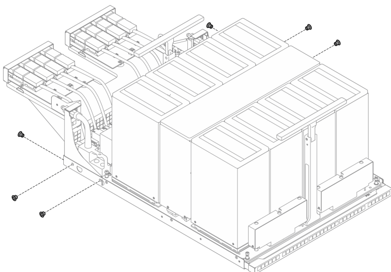
Figura 186. Rimozione delle viti
