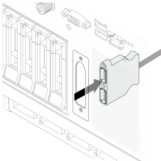
Figura 53. Rimozione dell'assieme USB
