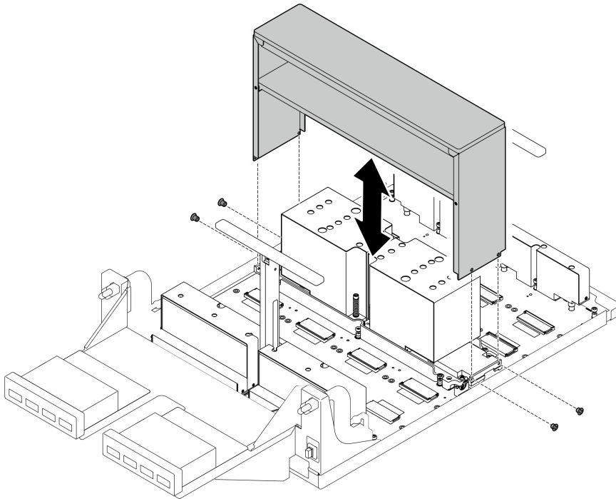
Figura 83. Rimozione del coperchio del dissipatore di calore NVSwitch
