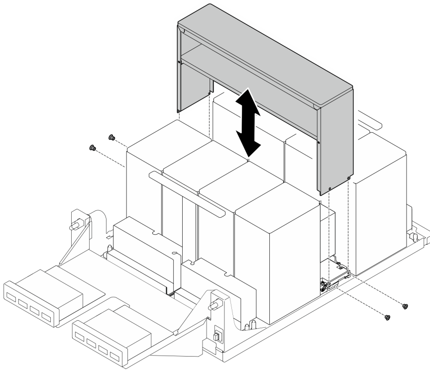
Figura 137. Rimozione del coperchio del dissipatore di calore NVSwitch
