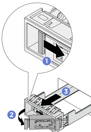
Figura 155. Rimozione del vassoio dell'unità M.2
