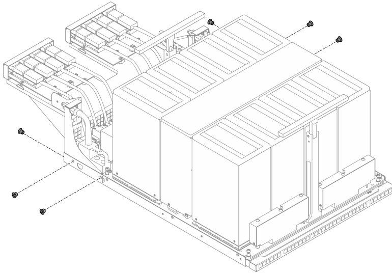
Figura 213. Installazione delle viti
