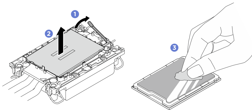
Figura 249. Separazione di un processore dal dissipatore di calore e dalla piastra
