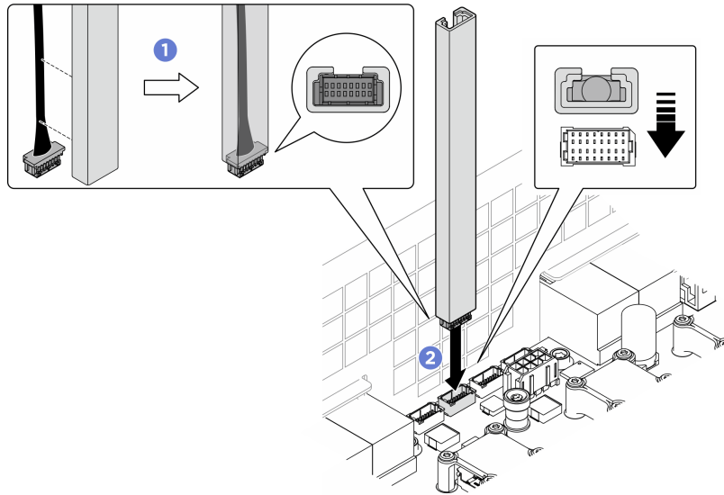
Figura 210. Installazione del cavo laterale
