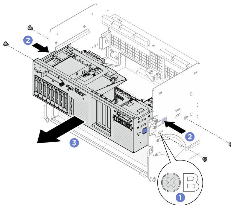
Figura 215. Trazione del telaio dell'unità NVMe e della scheda dello switch PCIe fino alla posizione di blocco
