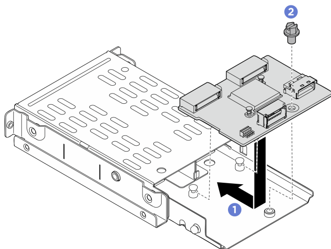
Figura 160. Installazione del backplane M.2
