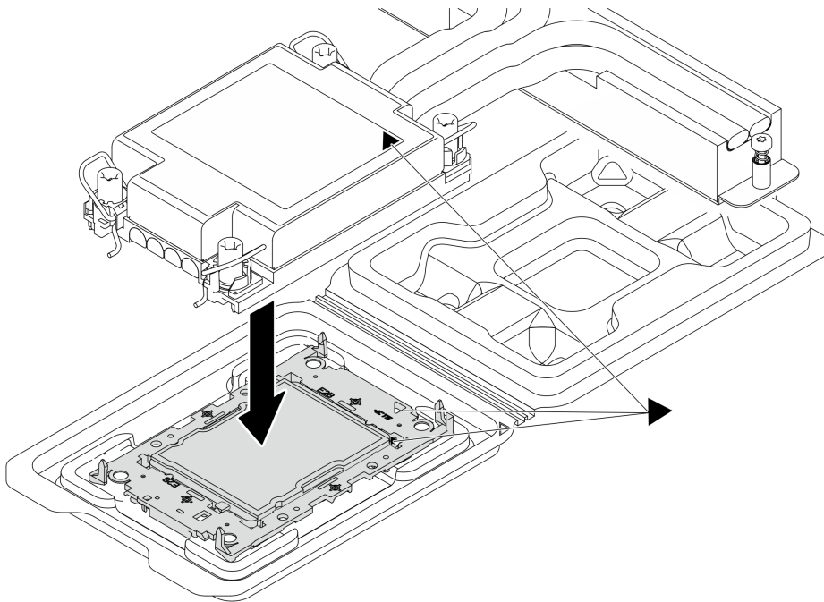
Figura 254. Assemblaggio del PHM con il processore nella confezione di spedizione
