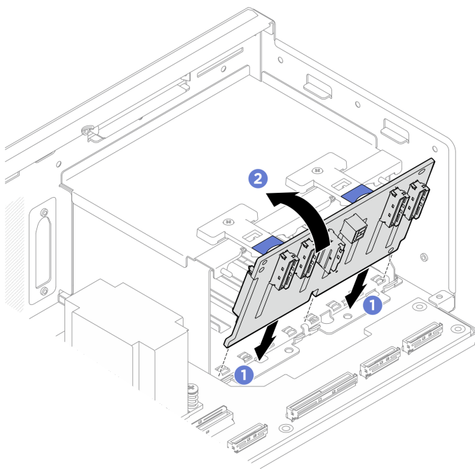
Figura 24. Installazione del backplane dell'unità da 2,5 pollici
