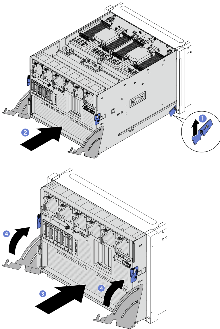
Figura 220. Installazione dello shuttle di sistema
