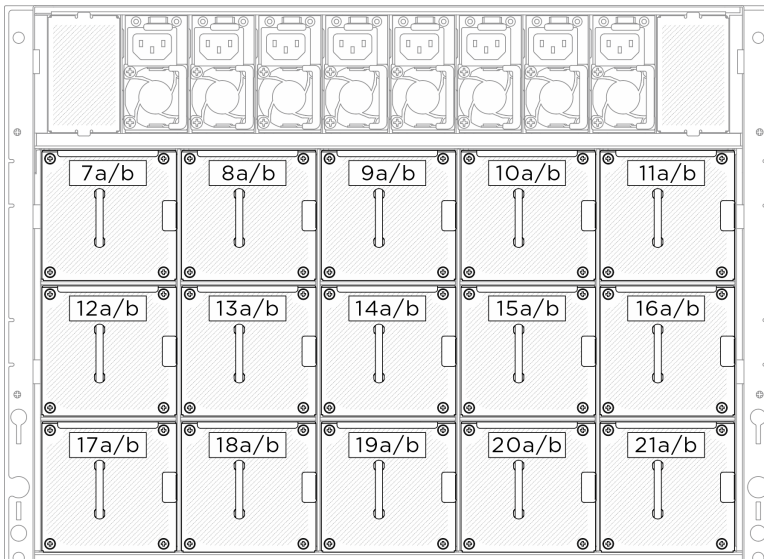
Figura 66. Numerazione delle ventole posteriori
