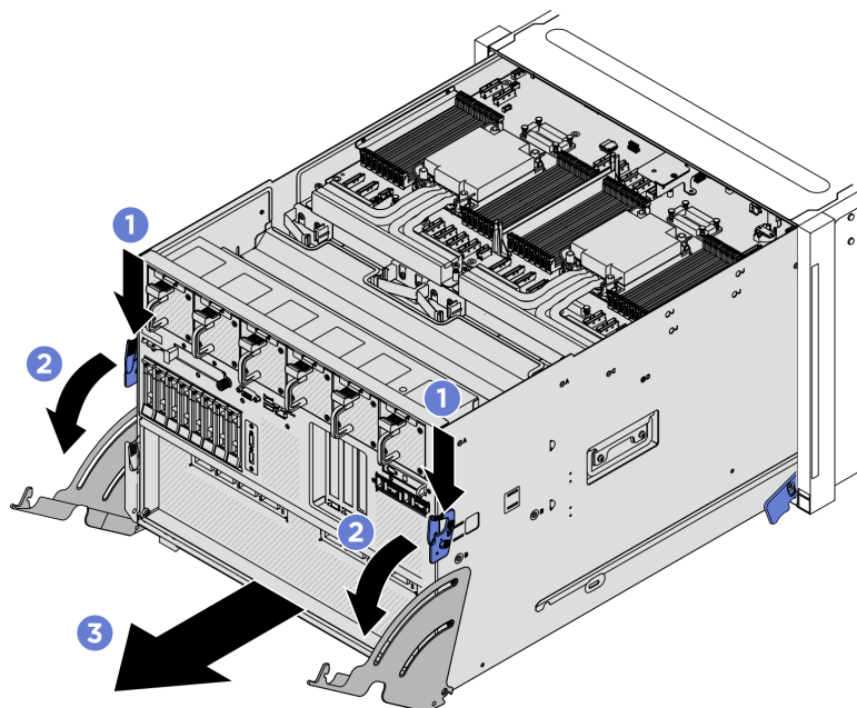
Figura 282. Trazione dello shuttle di sistema in posizione di arresto
