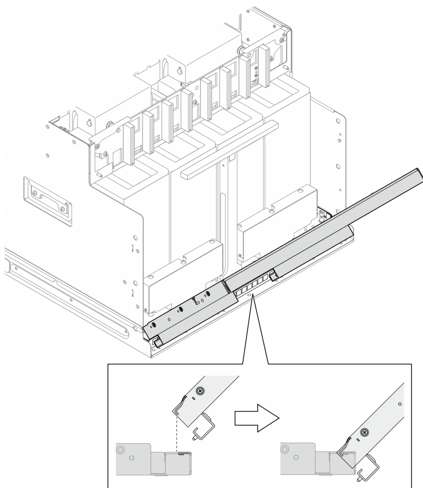
Figura 262. Aggancio della paratia della ventola posteriore alla staffa dello shuttle della GPU
