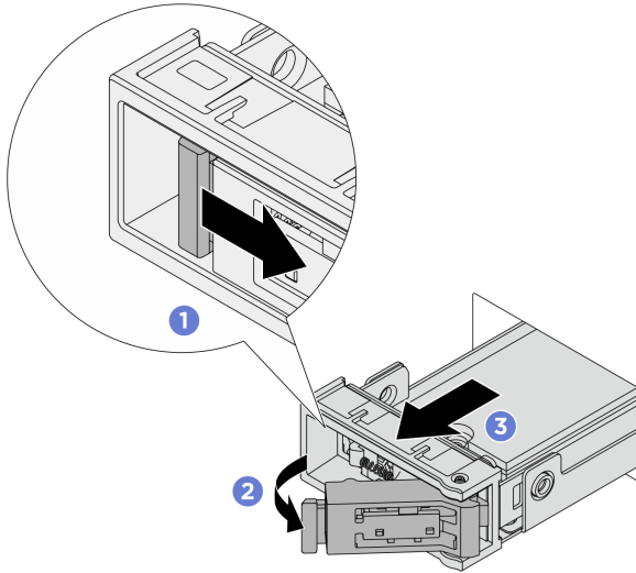
Figura 148. Rimozione dell'assieme dell'unità M.2 hot-swap
