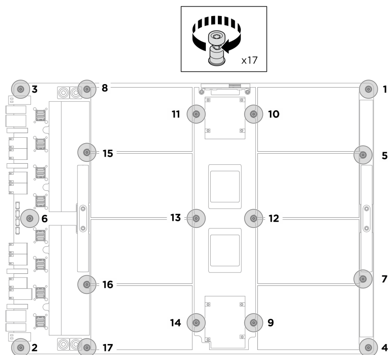
Figura 106. Installazione delle viti
