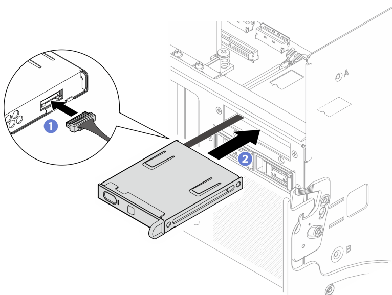
Figura 144. Installazione del pannello di diagnostica integrato
