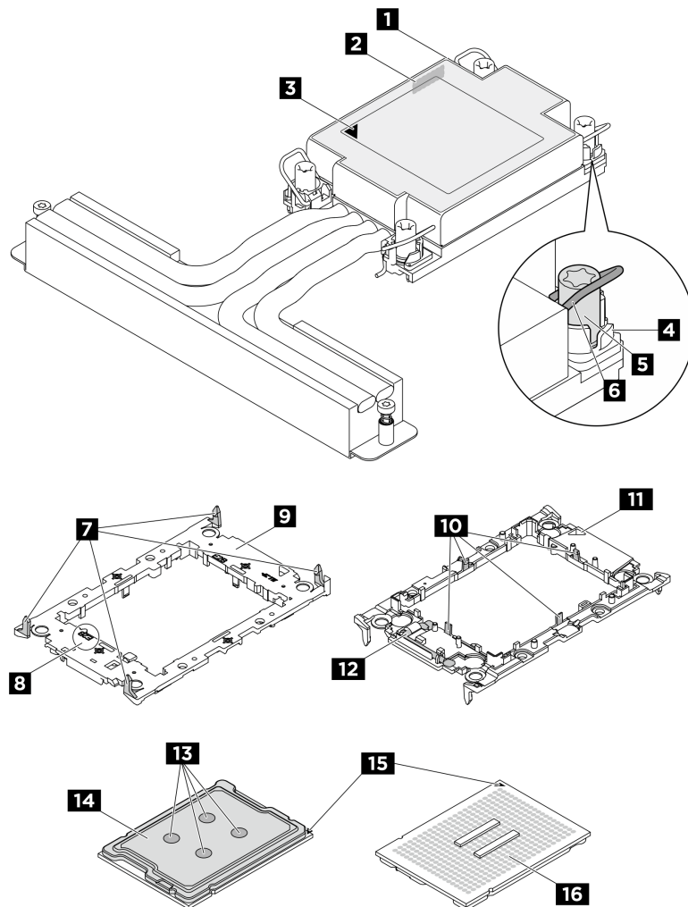
Figura 245. Componenti del PHM
