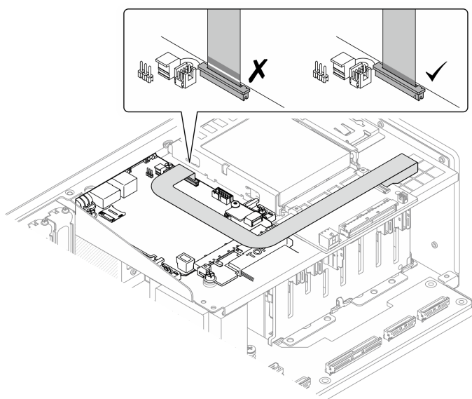
Figura 290. Ispezione dell'installazione del cavo FPC
