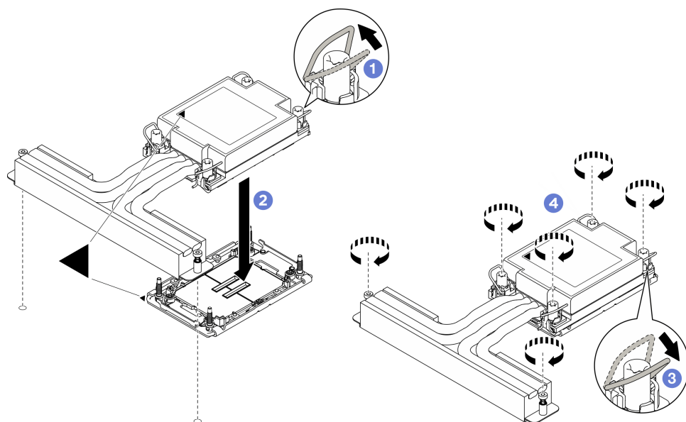
Figura 256. Installazione del PHM
