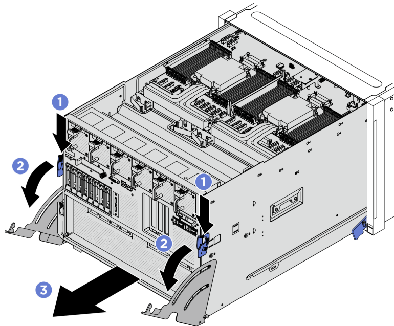
Figura 141. Trazione dello shuttle di sistema in posizione di arresto
