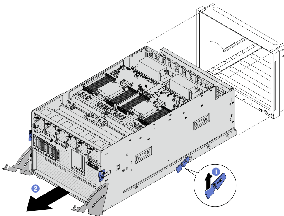
Figura 293. Rimozione dello shuttle di sistema
