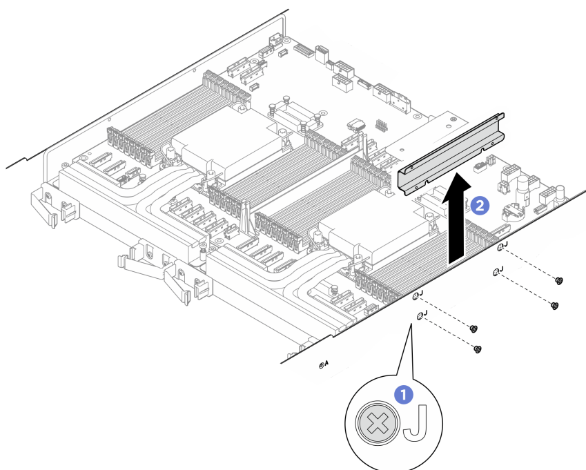
Figura 30. Rimozione della guida per il cavo destra
