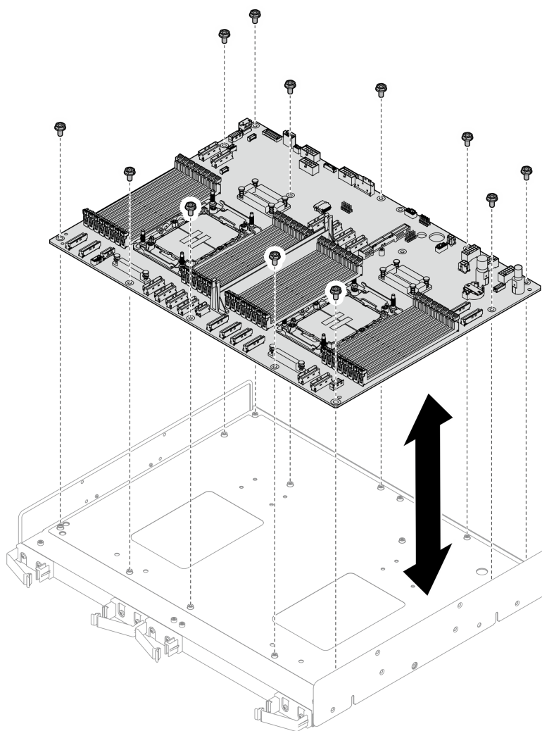
Figura 280. Rimozione della scheda di sistema
