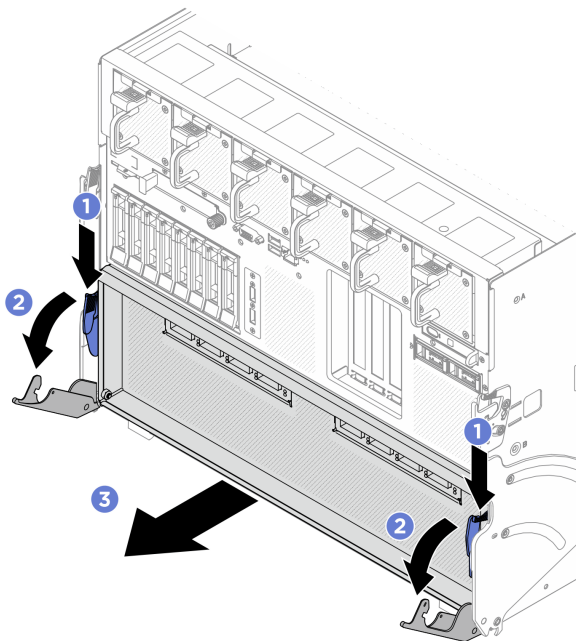
Figura 276. Sgancio dello shuttle della scheda retimer
