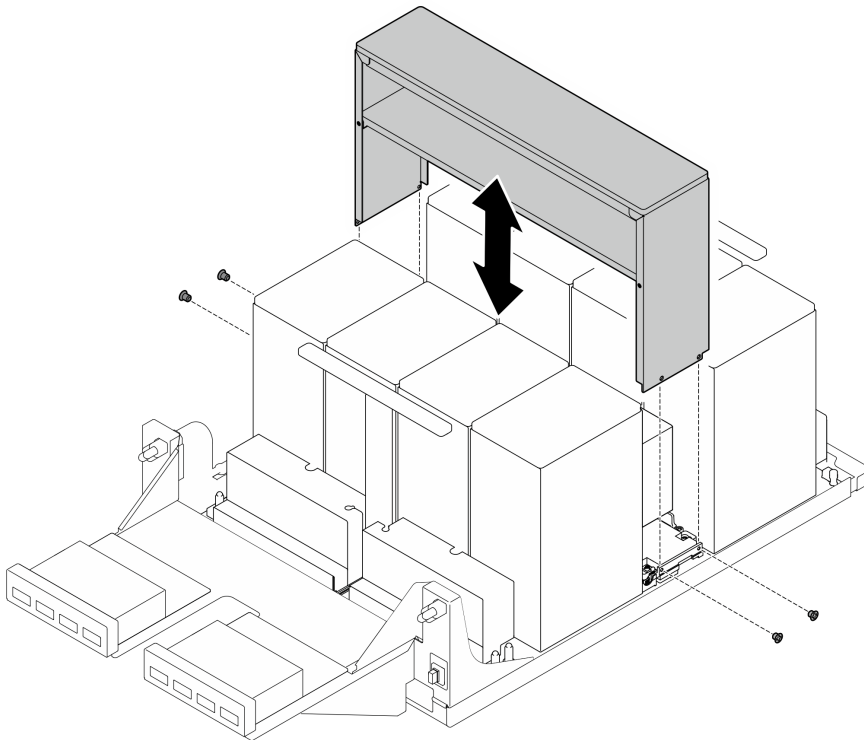
Figura 99. Rimozione del coperchio del dissipatore di calore NVSwitch
