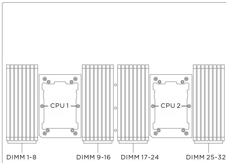
Figura 165. Layout dei moduli di memoria e dei processori
