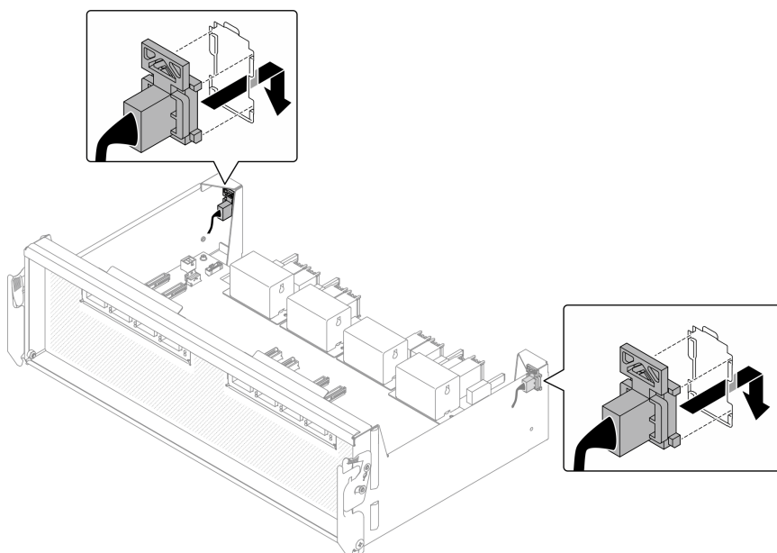
Figura 273. Installazione del cavo laterale della scheda OSFP
