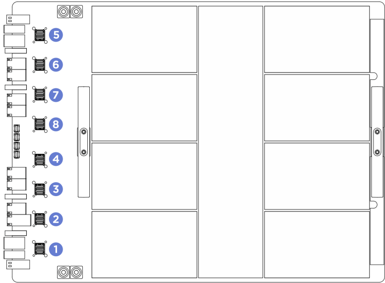
Figura 202. Sequenza di installazione dei cavi UltraPass
