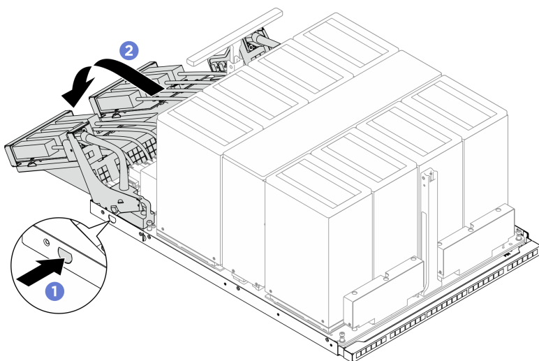
Figura 187. Sgancio del vassoio di supporto OSFP
