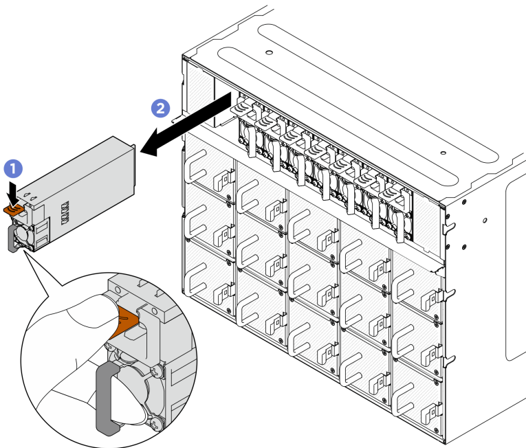
Figura 240. Rimozione dell'unità di alimentazione
