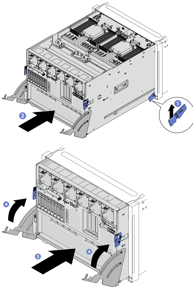
Figura 258. Installazione dello shuttle di sistema
