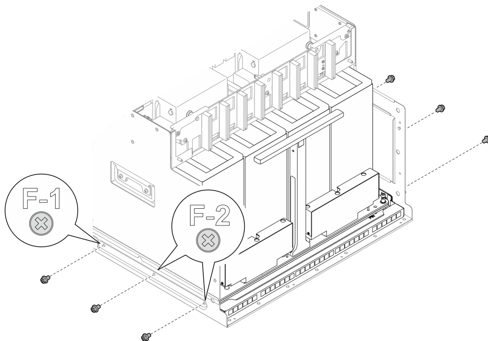
Figura 119. Rimozione delle viti
