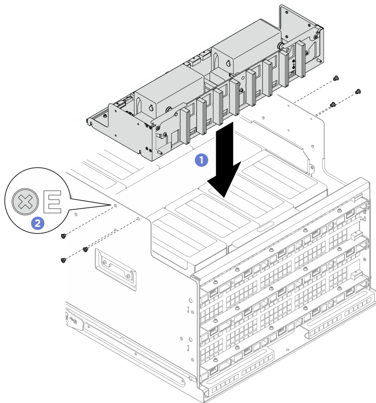
Figura 236. Installazione del complesso di alimentazione
