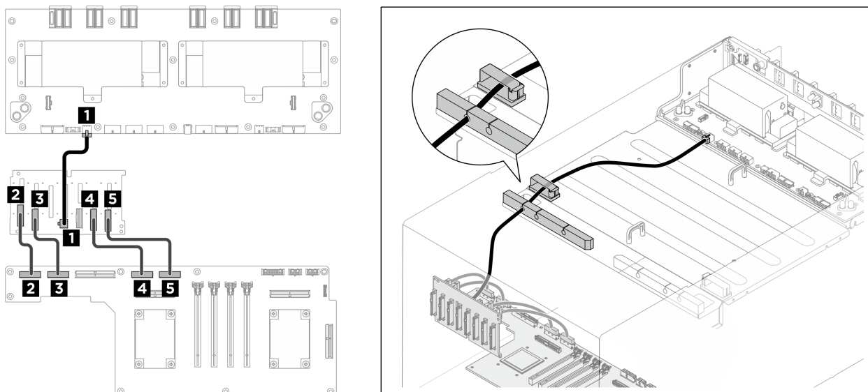
Figura 310. Instradamento dei cavi del backplane 1
