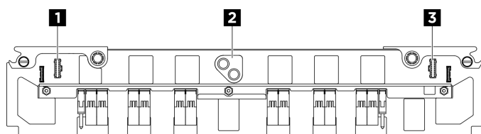
Figura 305. Connettori dell'interposer PSU
