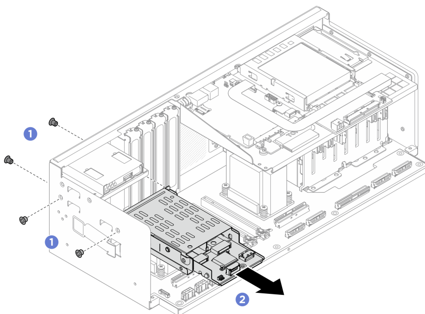
Figura 158. Rimozione del telaio dell'unità M.2
