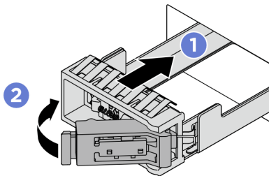
Figura 149. Installazione di un vassoio dell'unità M.2
