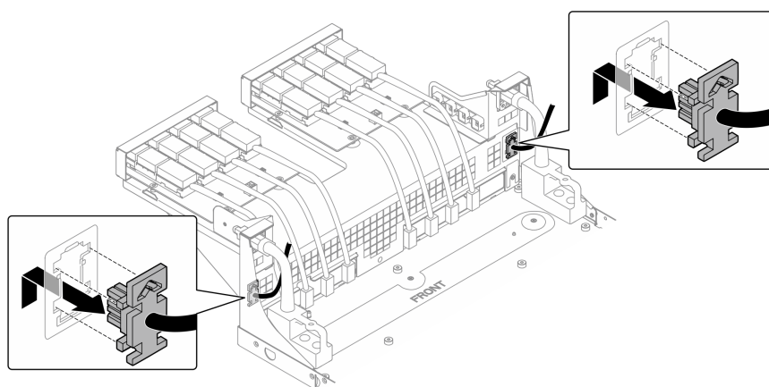
Figura 123. Rimozione del cavo laterale della scheda OSFP
