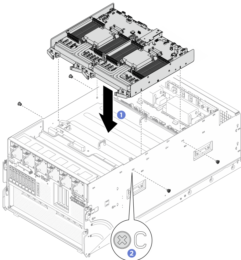
Figura 40. Installazione del vassoio di elaborazione
