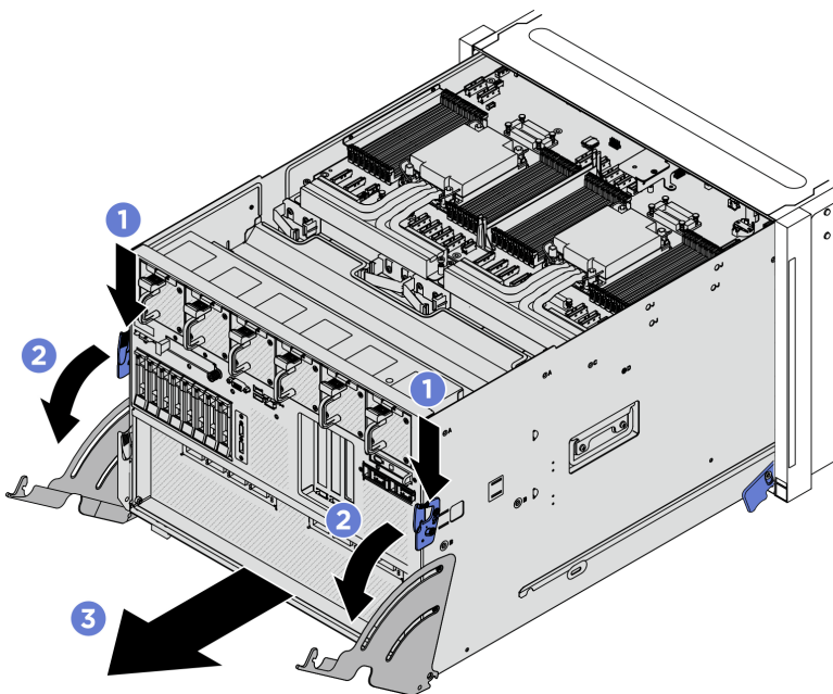
Figura 48. Trazione dello shuttle di sistema in posizione di arresto
