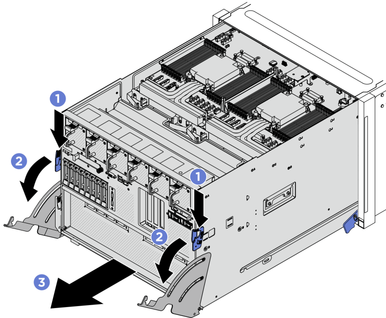
Figura 292. Trazione dello shuttle di sistema in posizione di arresto
