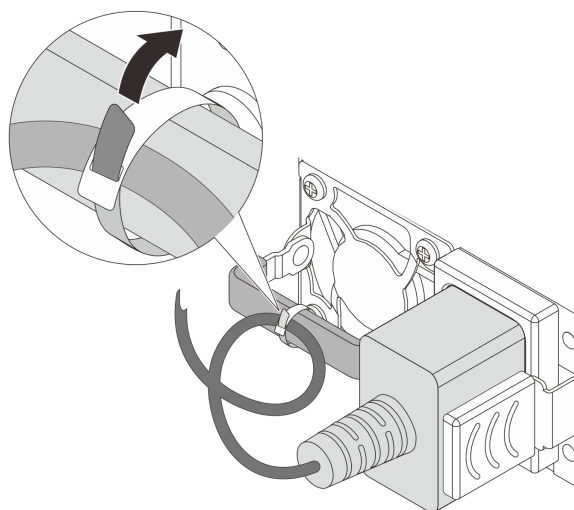
Figura 243. Instradamento e legatura del cavo di alimentazione
