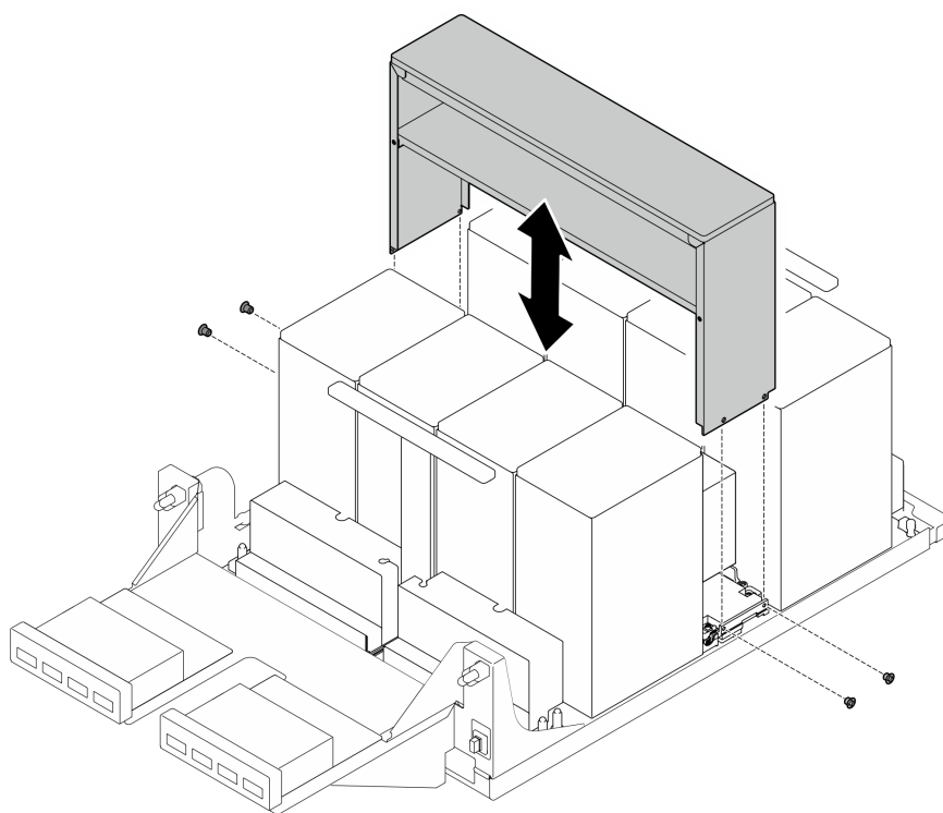
Figura 136. Installazione del coperchio del dissipatore di calore NVSwitch
