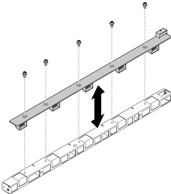
Figura 76. Installazione della scheda di controllo della ventola posteriore
