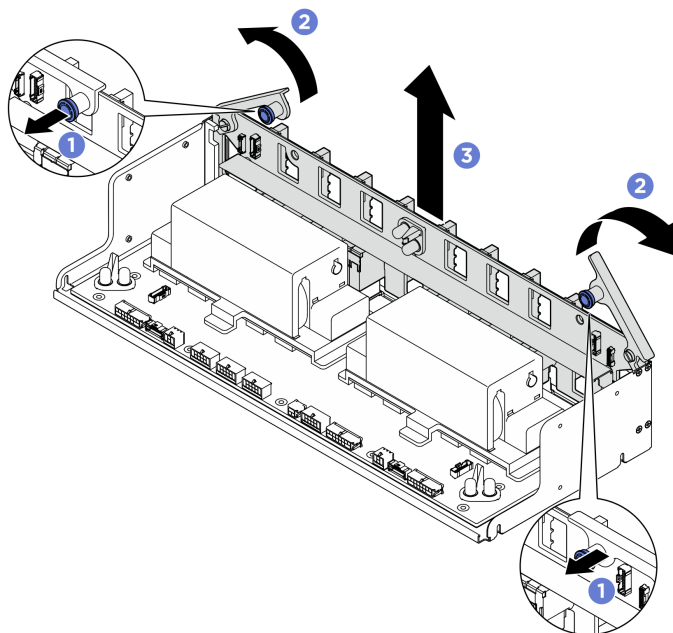
Figura 259. Rimozione dell'interposer PSU
