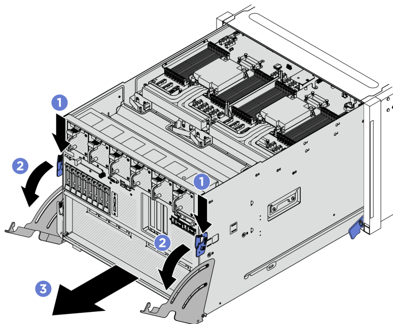
Figura 246. Trazione dello shuttle di sistema in posizione di arresto
