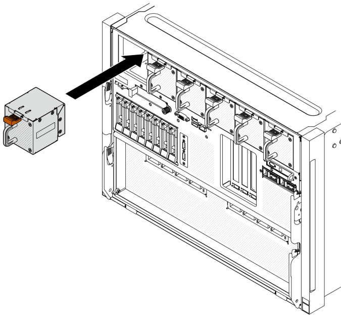
Figura 67. Installazione della ventola anteriore
