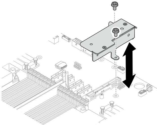
Figura 31. Rimozione della guida per il cavo centrale
