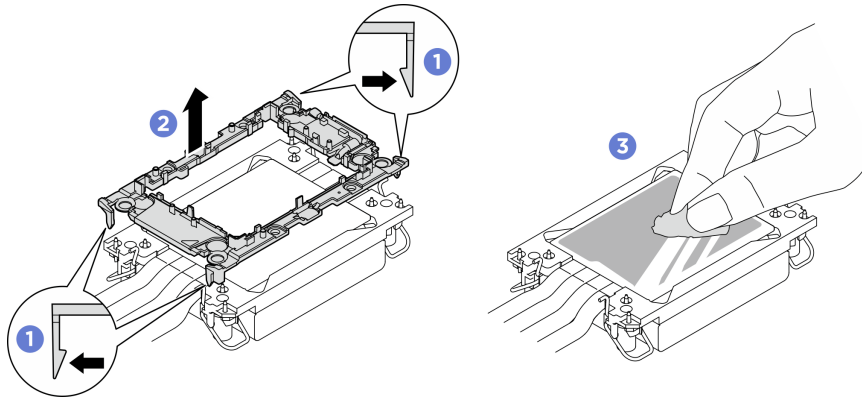
Figura 250. Separazione di una piastra del processore dal dissipatore di calore
