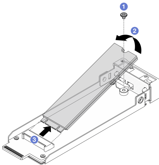
Figura 150. Rimozione dell'unità M.2
