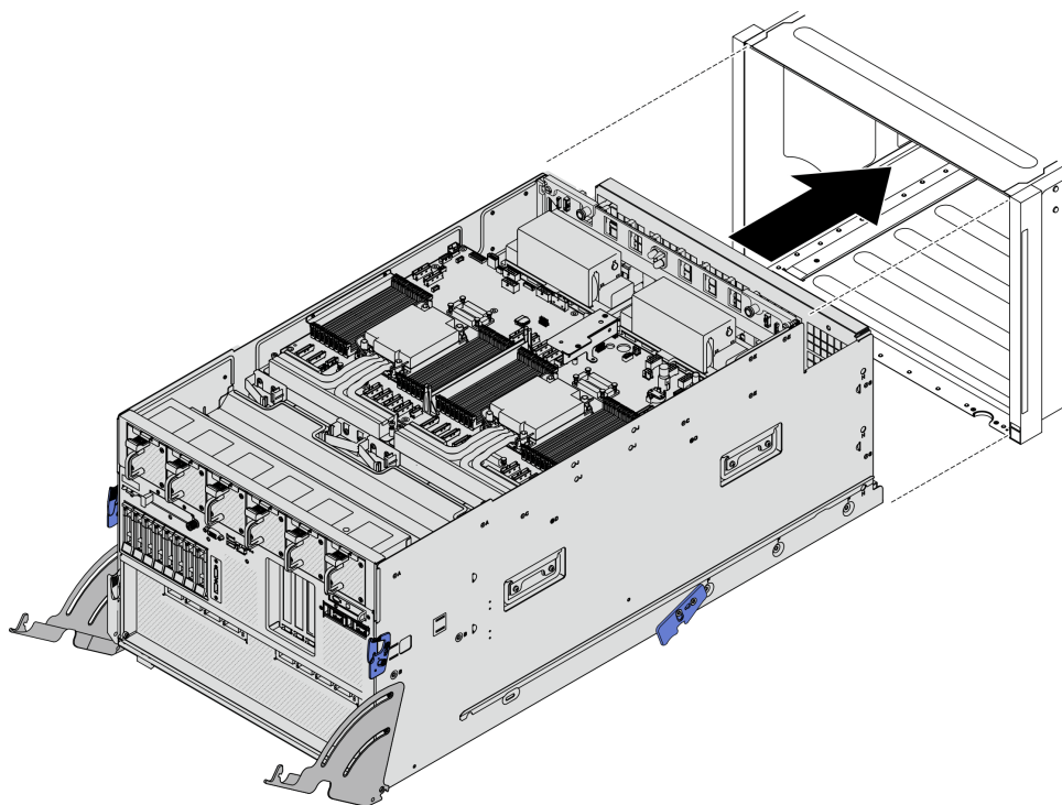
Figura 294. Spingere lo shuttle di sistema in posizione di arresto
