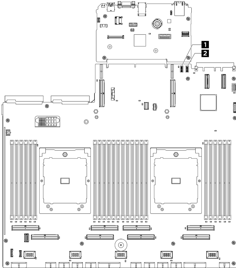
Figura 12. Switch dell'assieme della scheda di sistema
