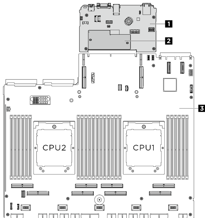
Figura 10. Layout dell'assieme della scheda di sistema
