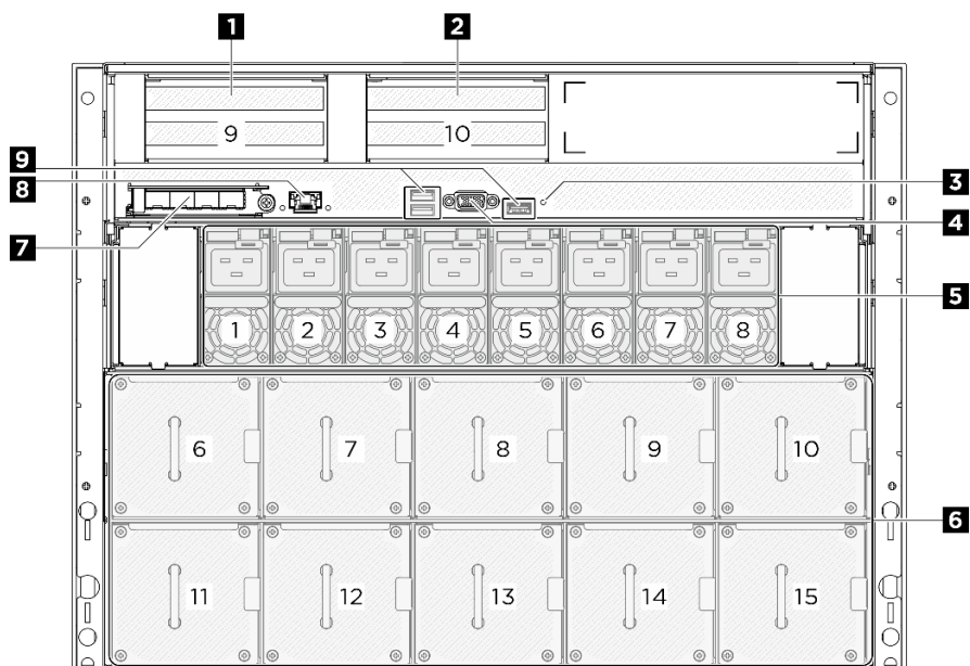
Figura 4. Vista posteriore
