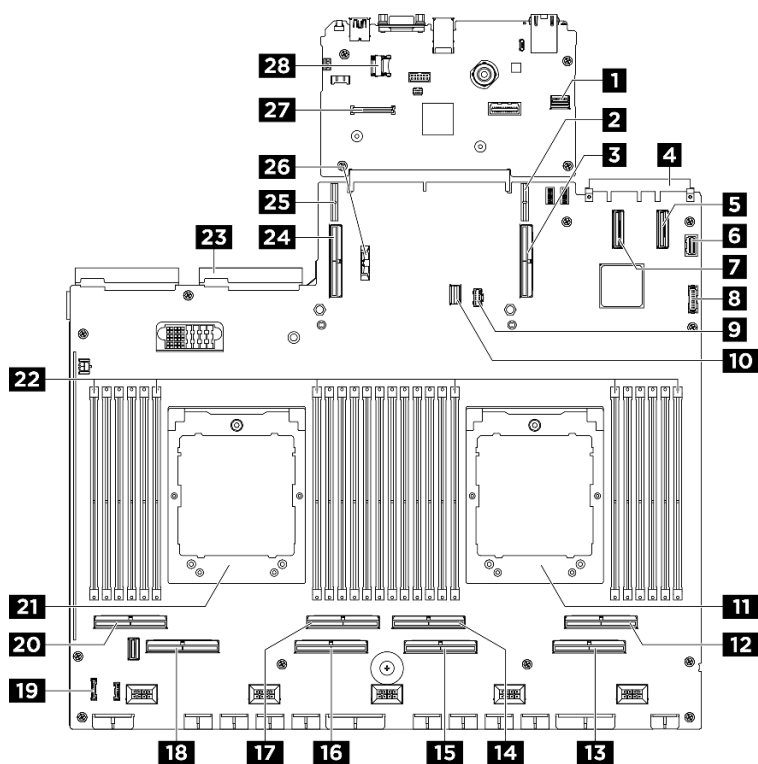
Figura 11. Connettori sull'assieme della scheda di sistema
