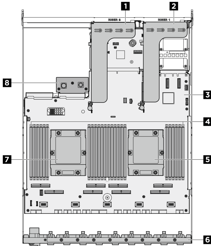
Figura 7. Vista superiore dello shuttle di elaborazione 2U
