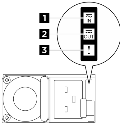
Figura 14. LED dell'alimentatore CFFv4
