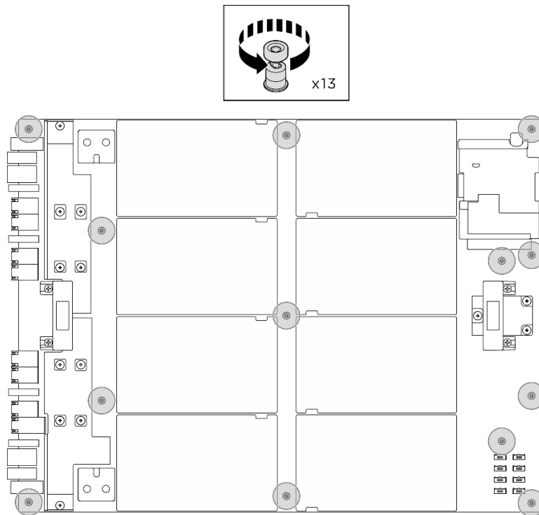
Figura 82. Remoção do parafuso
