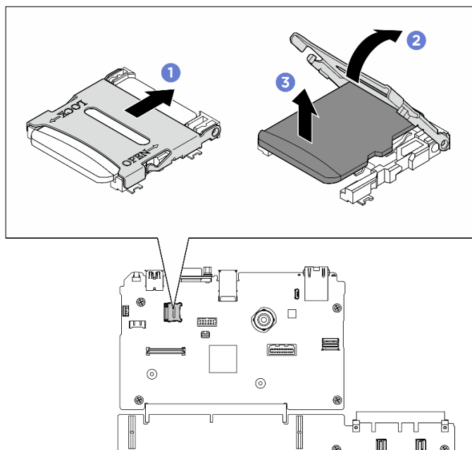
Figura 122. Remoção do cartão microSD
