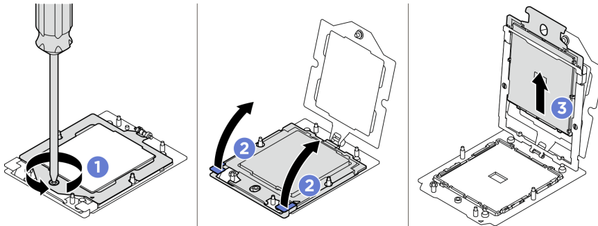
Figura 185. Remoção do processador
