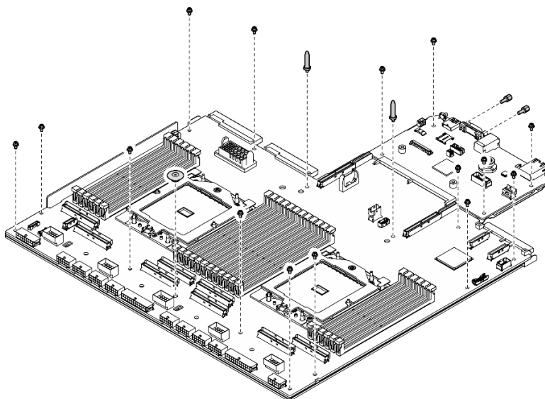
Figura 206. Remoção do componente
