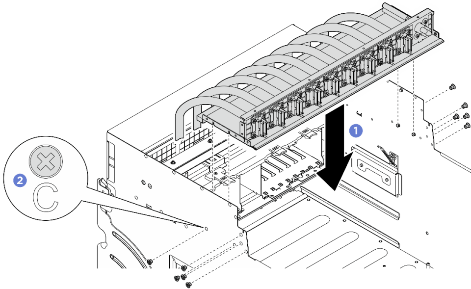
Figura 155. Instalação do Conjunto de cabos do comutador PCIe frontal
