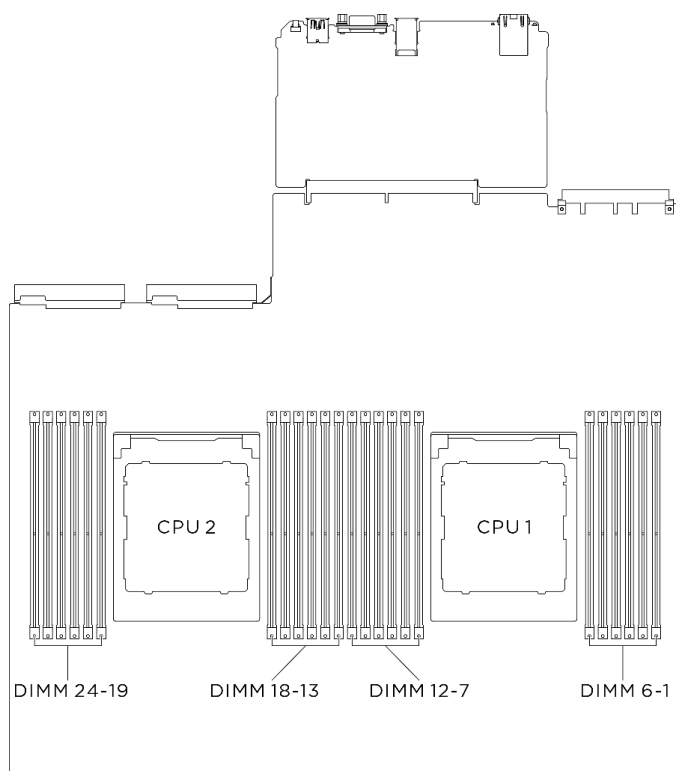
Figura 120. Layout de módulos de memória e processadores
