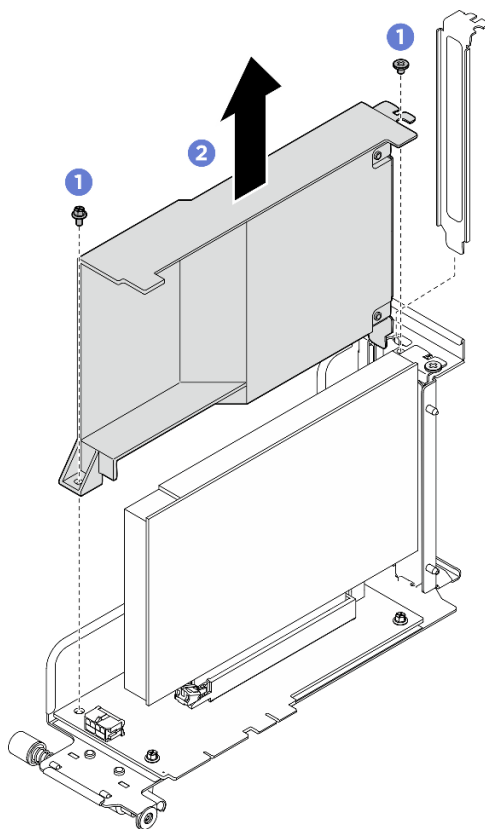
Figura 132. Remoção do defletor de ar da placa riser PCIe
