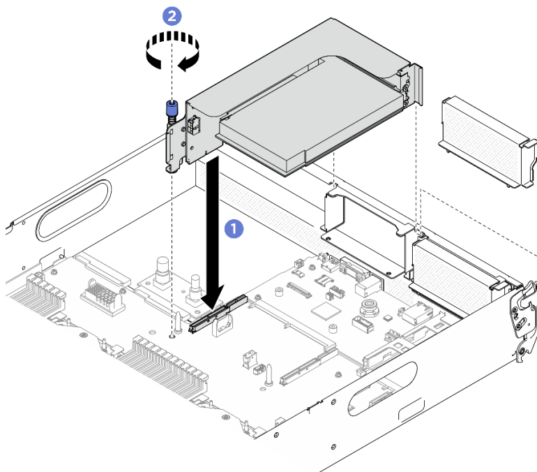
Figura 141. Instalação do conjunto de placa riser PCIe
