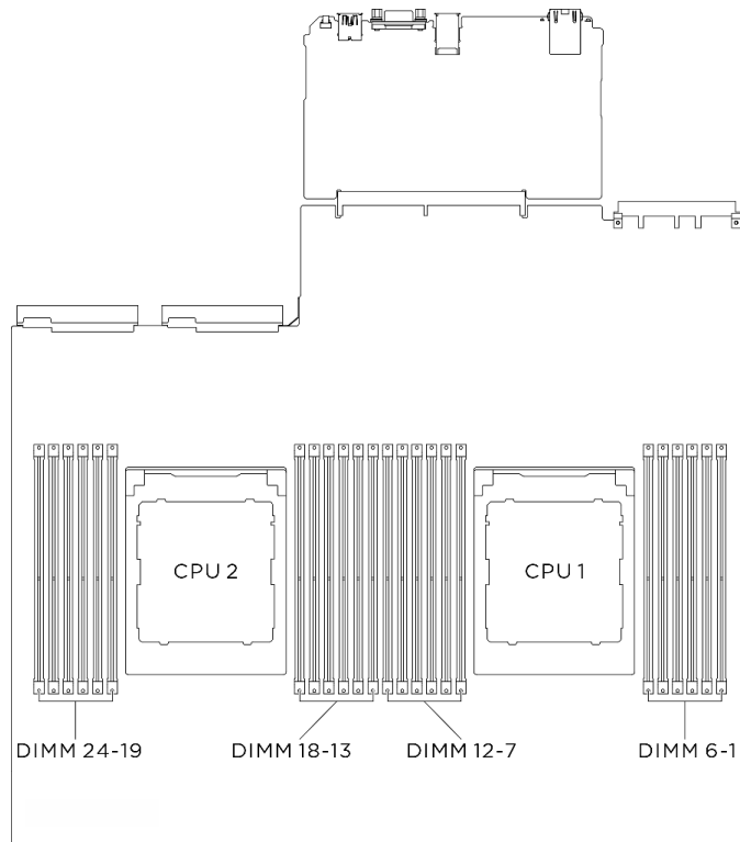
Figura 1. Layout de módulos de memória e processadores
