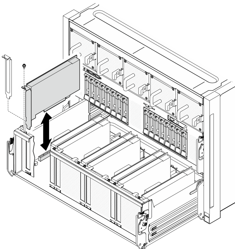
Figura 128. Instalação do adaptador PCIe frontal
