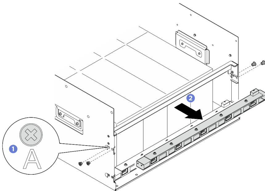
Figura 45. Remoção do conjunto de placa de controle do ventilador traseiro
