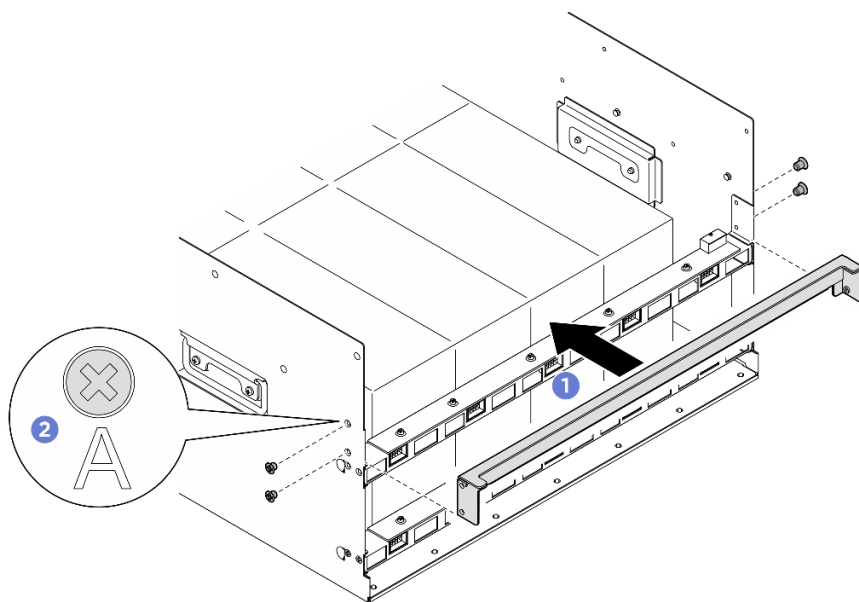
Figura 87. Instalação do suporte de apoio traseiro
