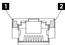
Figura 253. LEDs da Porta de gerenciamento de sistemas XCC (10/100/1.000 Mbps RJ-45)
