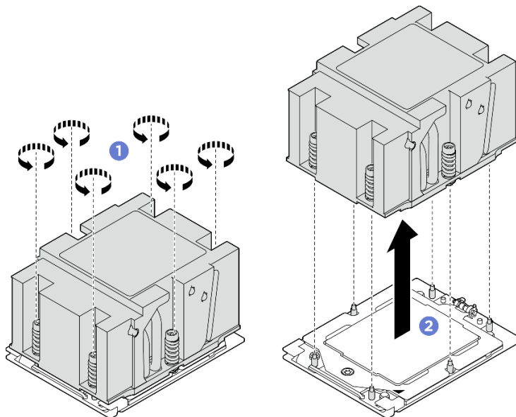
Figura 184. Remoção do dissipador de calor
