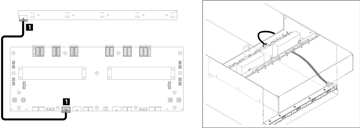
Figura 235. Roteamento de cabos da placa de controle do ventilador traseiro (inferior)
