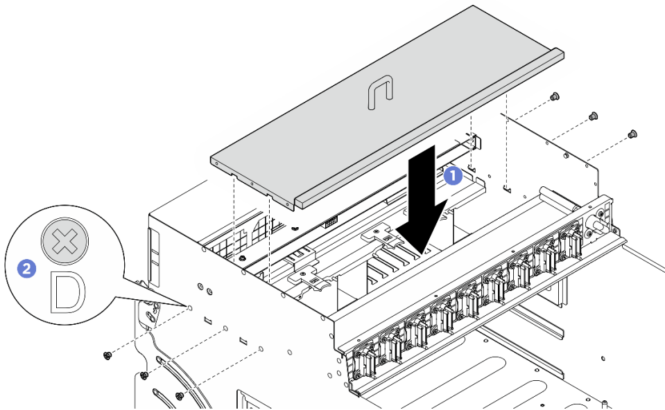
Figura 108. Instalação da tampa de E/S
