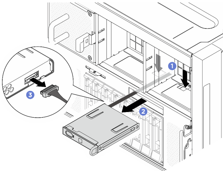
Figura 105. Remoção do painel de diagnóstico integrado
