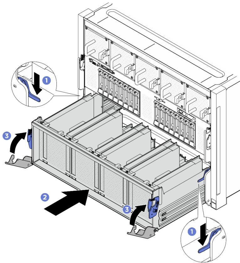
Figura 66. Instalação do Alternador do comutador PCIe no Alternador de GPU 8U
