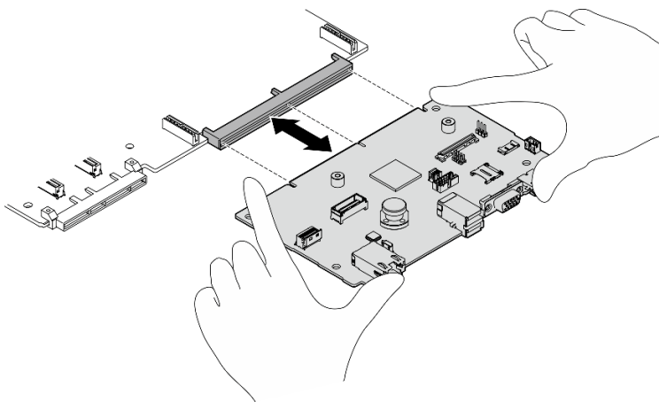
Figura 209. Instalação da placa de E/S do sistema
