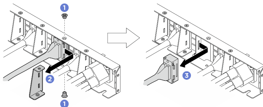
Figura 159. Remoção do módulo de E/S frontal, do painel de diagnóstico integrado, do gerenciamento de GPU ou do cabo de sinal
