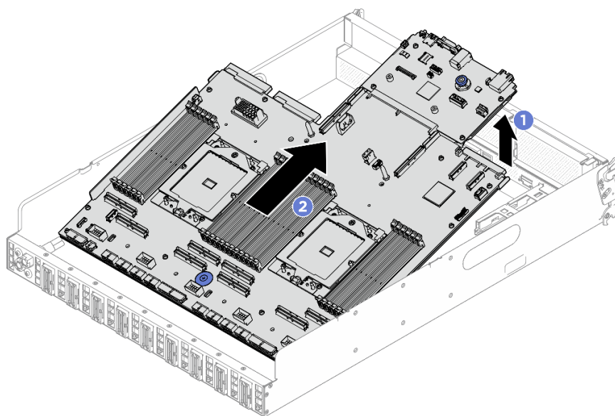
Figura 202. Remoção do conjunto de placa-mãe
