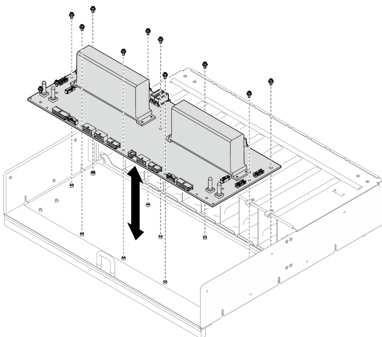
Figura 172. Instalação da placa de distribuição de energia
