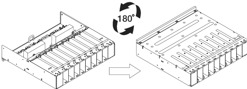
Figura 50. Virando o complexo de energia para baixo
