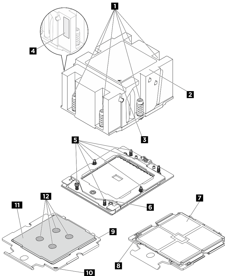
Figura 183. Componentes do processador e do dissipador de calor
