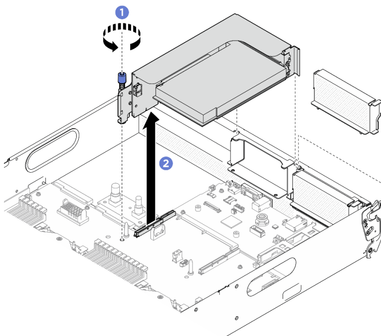
Figura 135. Remoção do conjunto de placa riser PCIe
