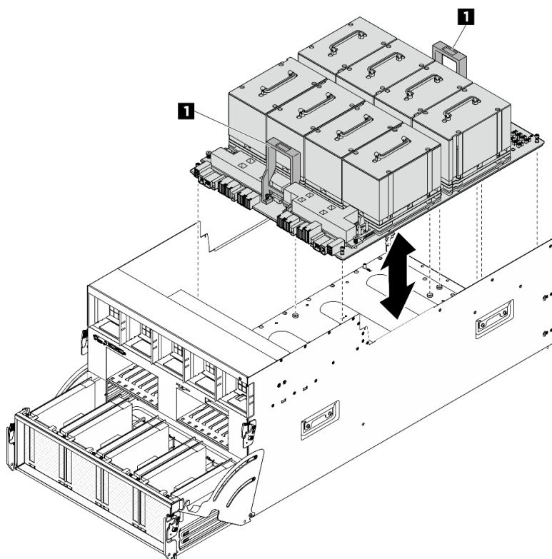
Figura 83. Remoção do Complexo da GPU
