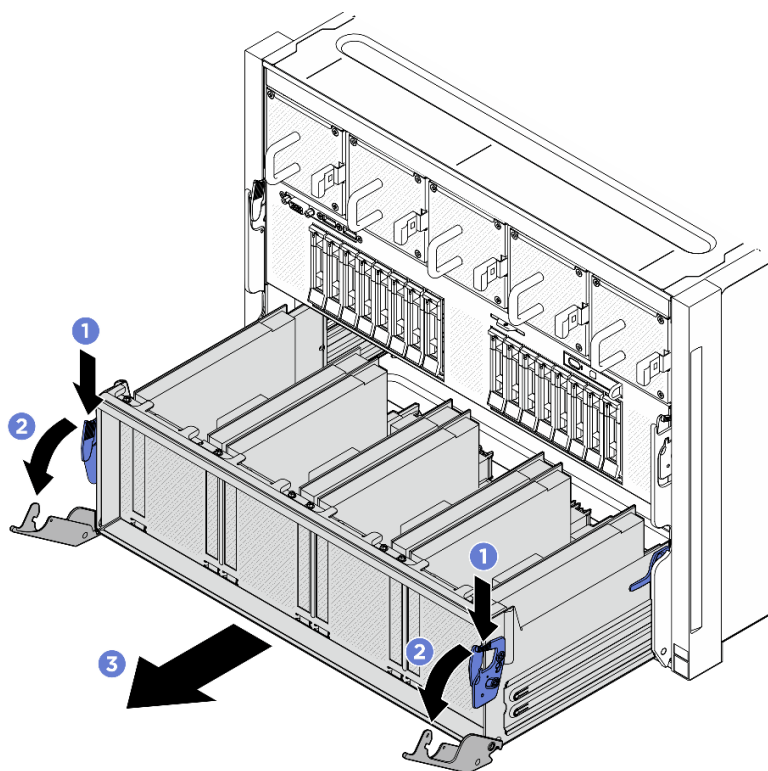
Figura 89. Remoção do Alternador do comutador PCIe para a posição de parada
