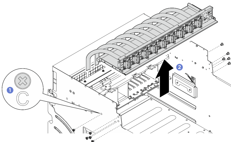
Figura 149. Remoção do Conjunto de cabos do comutador PCIe frontal
