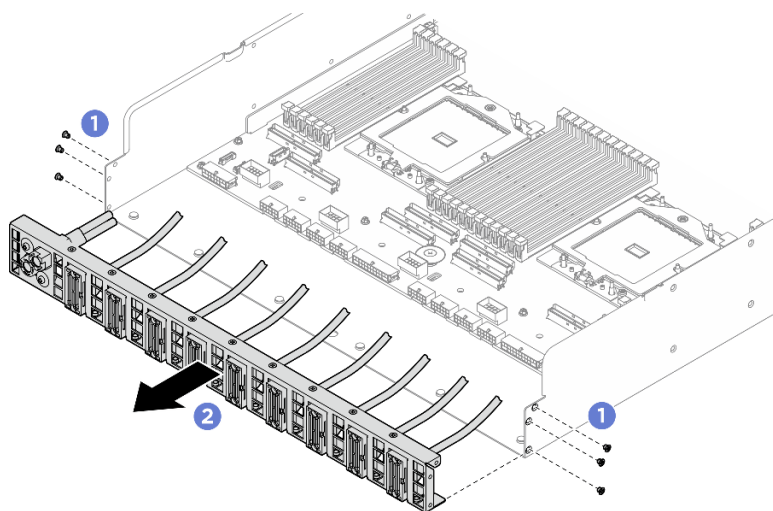
Figura 158. Remoção do Conjunto de cabos do comutador PCIe traseiro
