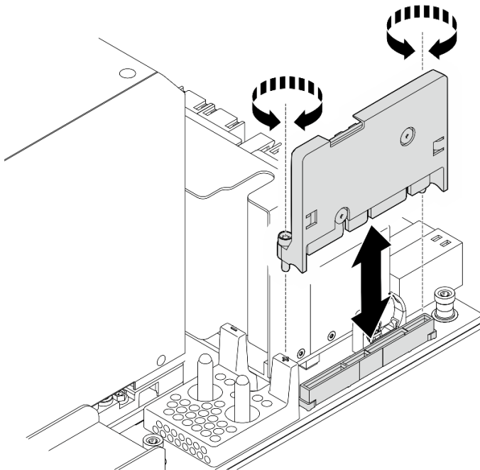
Figura 103. Remoção da placa HMC
