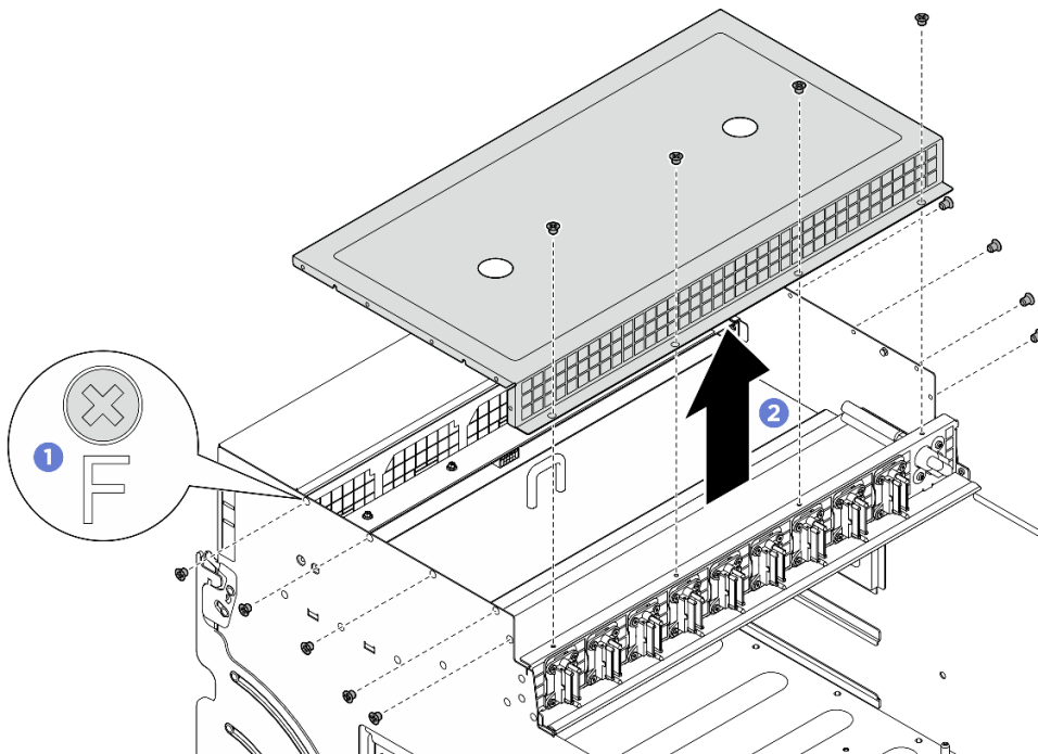
Figura 30. Remoção da tampa do cabo
