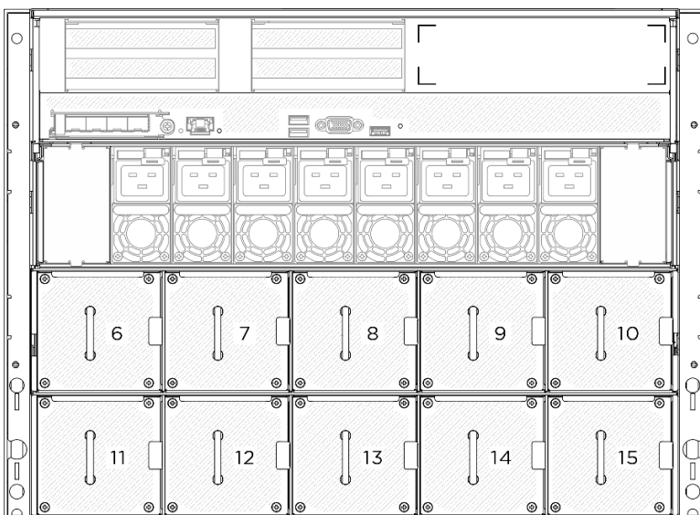
Figura 35. Numeração do ventilador traseiro
