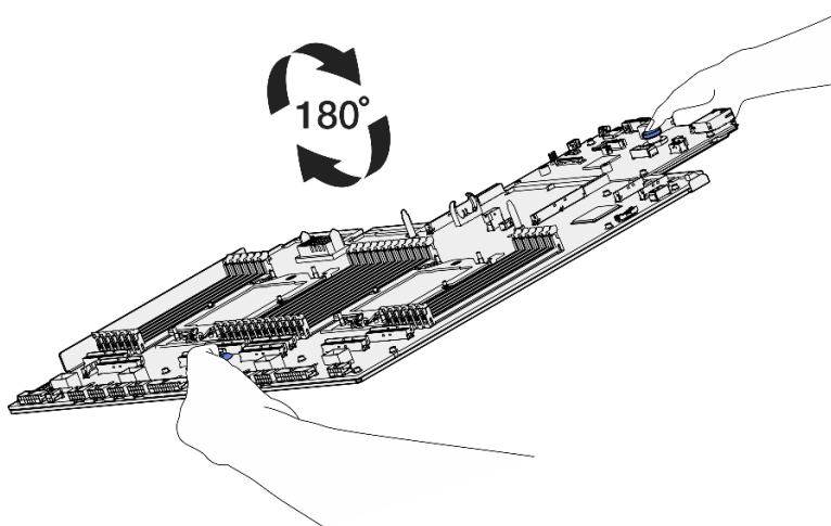
Figura 203. Girando o conjunto de placa-mãe para baixo
