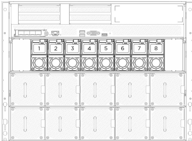
Figura 176. Numeração do preenchimento do compartimento de fonte de alimentação
