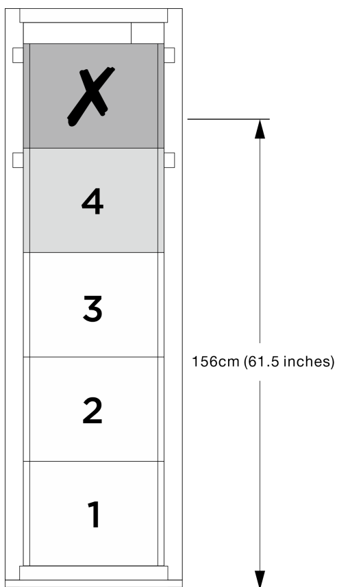
Figura 9. Altura máxima de instalação
