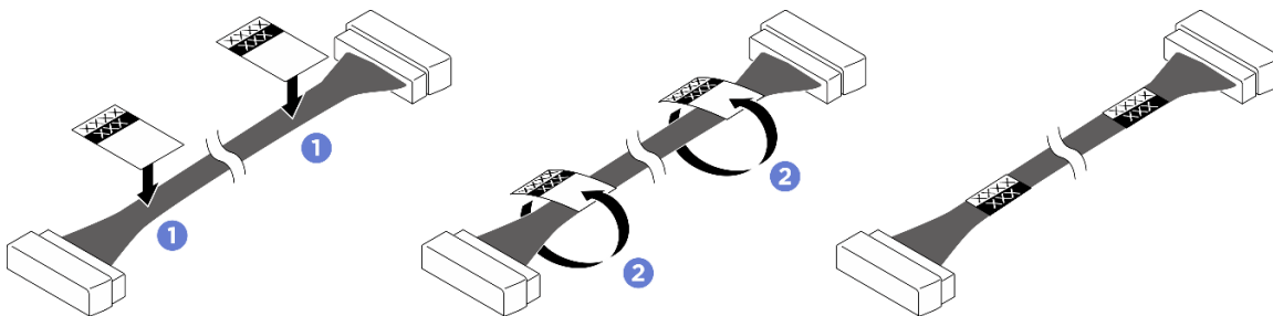
Figura 25. Aplicação de etiqueta
