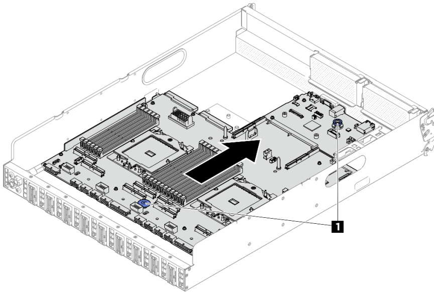
Figura 216. Instalação do conjunto de placa-mãe
