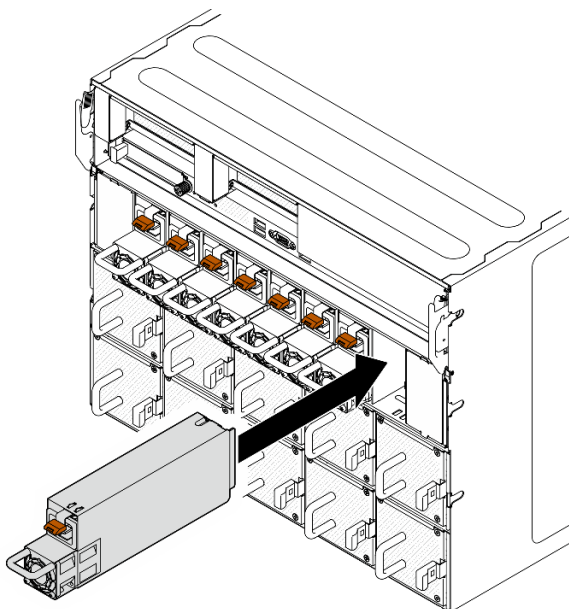
Figura 179. Instalação da unidade de fonte de alimentação
