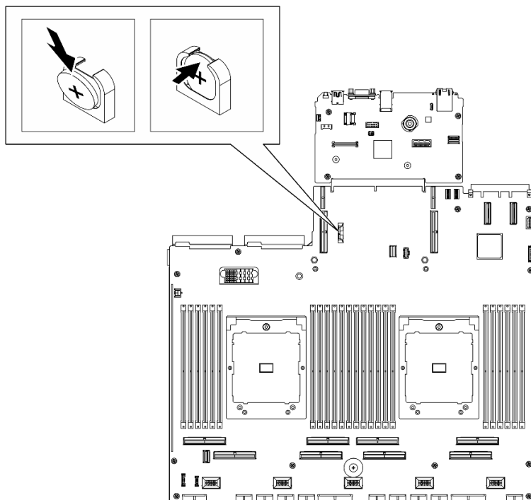
Figura 33. Instalação da bateria CMOS
