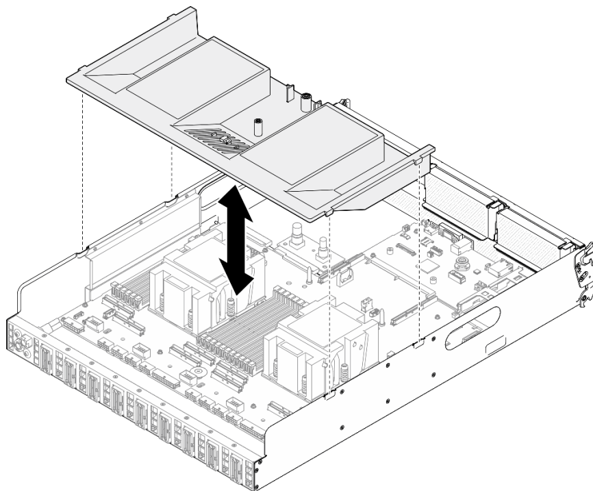
Figura 181. Instalação do defletor de ar do processador
