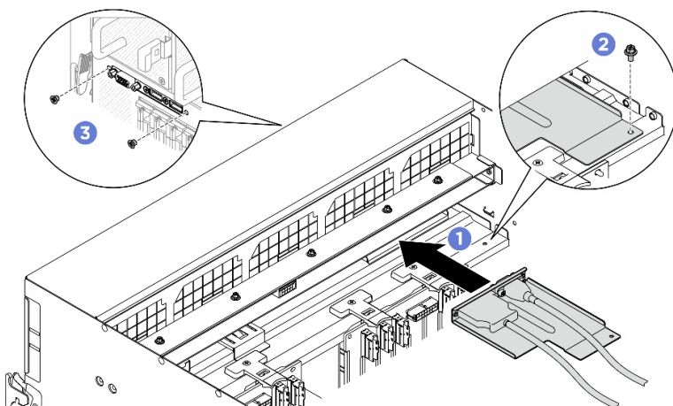
Figura 157. Instalação do módulo de E/S frontal
