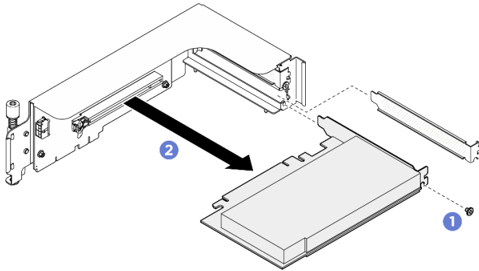
Figura 130. Remoção do adaptador PCIe traseiro
