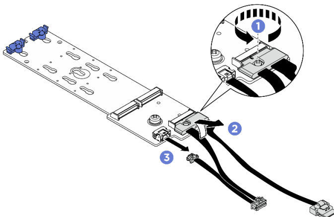
Figura 111. Desconexão do cabo do backplane M.2
