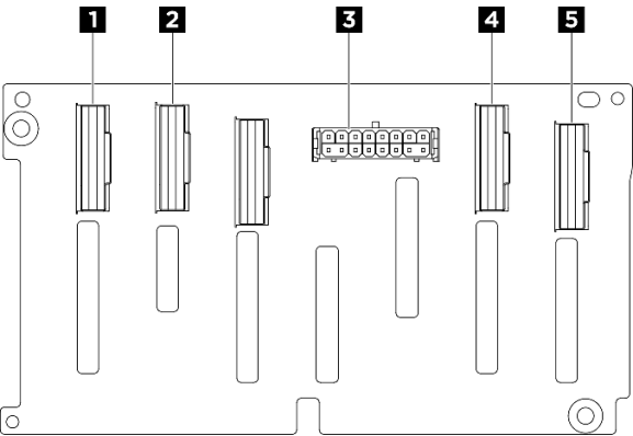
Figura 218. Conectores do backplane NVMe de 2,5 polegadas
