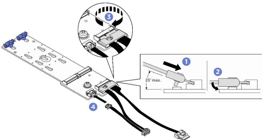
Figura 112. Conexão do cabo do backplane M.2
