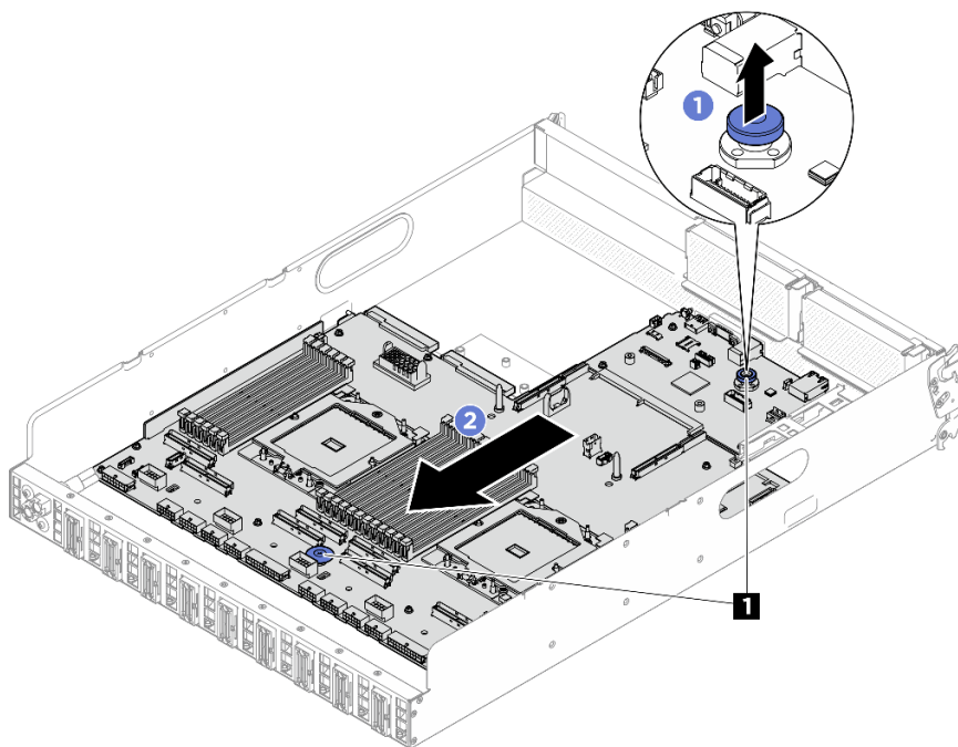
Figura 201. Desencaixe do conjunto da placa-mãe
