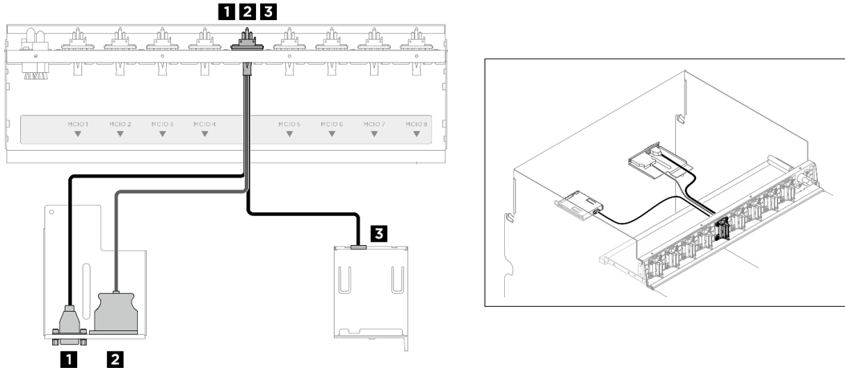
Figura 238. Roteamento de cabos do módulo de E/S frontal e do painel de diagnóstico integrado
