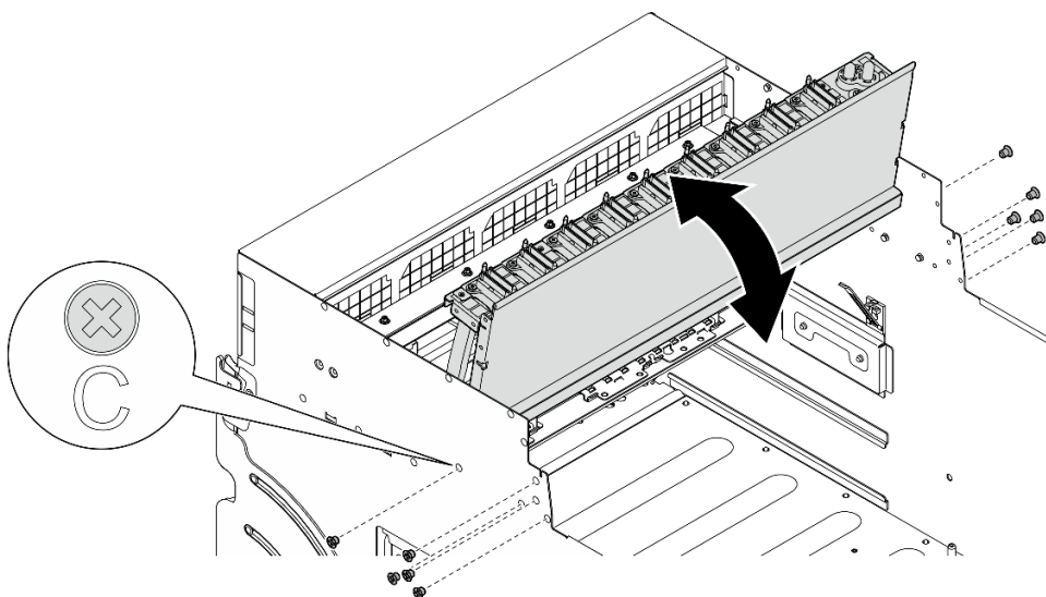
Figura 59. Virando o conjunto de cabos do comutador PCIe frontal
