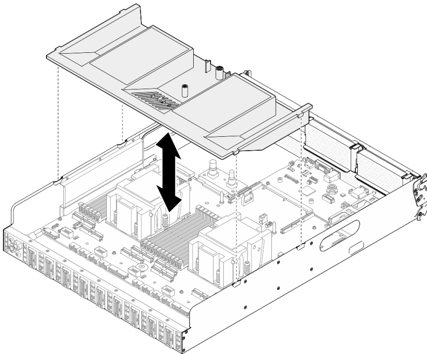
Figura 180. Remoção do defletor de ar do processador
