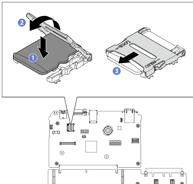
Figura 123. Instalação do cartão microSD
