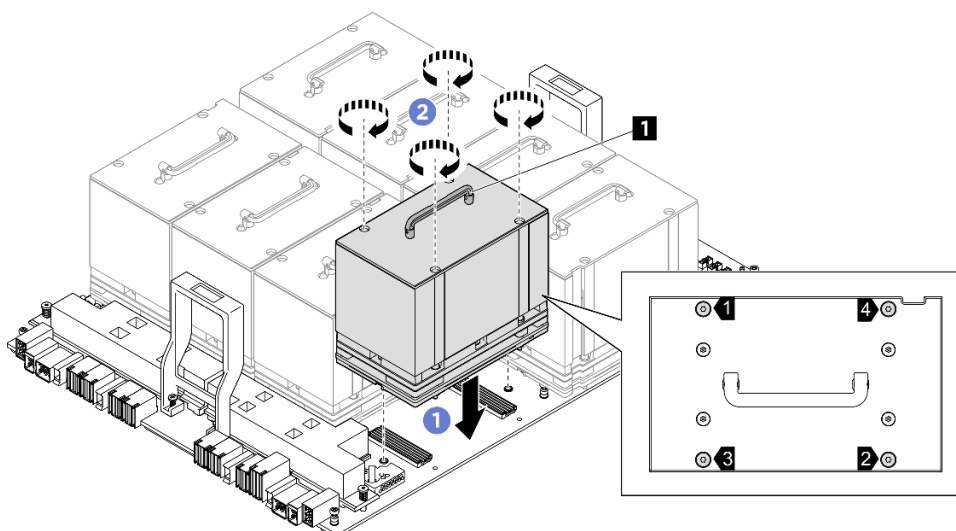
Figura 102. Instalação do Módulo de GPU e dissipador de calor
