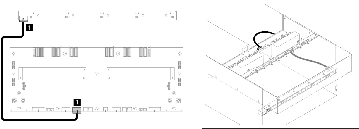
Figura 234. Roteamento de cabos da placa de controle do ventilador traseiro (superior)
