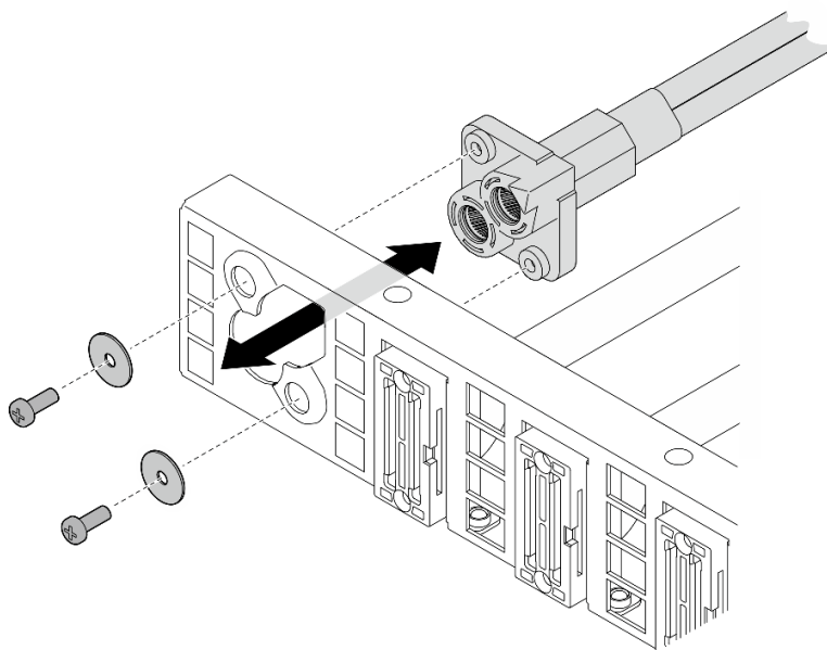
Figura 162. Instalação do cabo de alimentação
