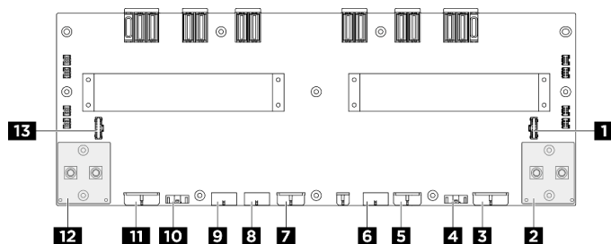
Figura 225. Conectores da placa de distribuição de energia
