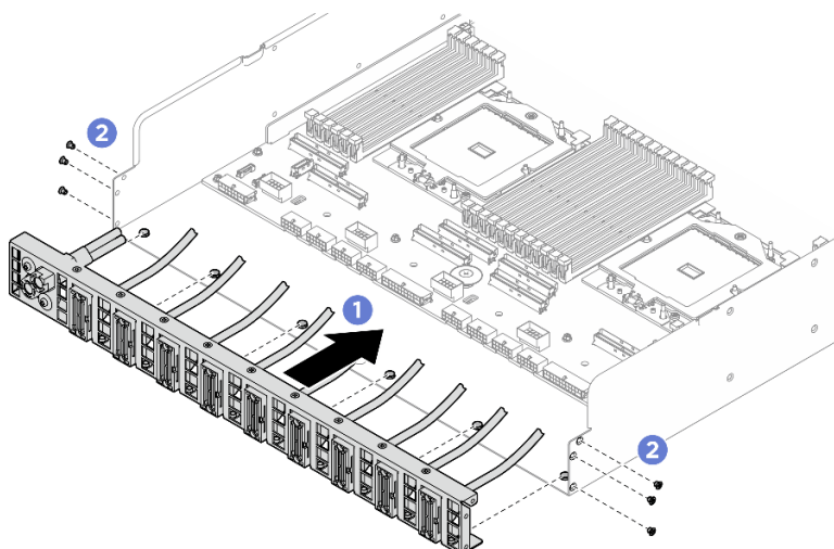
Figura 163. Instalação do Conjunto de cabos do comutador PCIe traseiro
