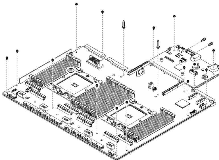
Figura 211. Instalação de componentes
