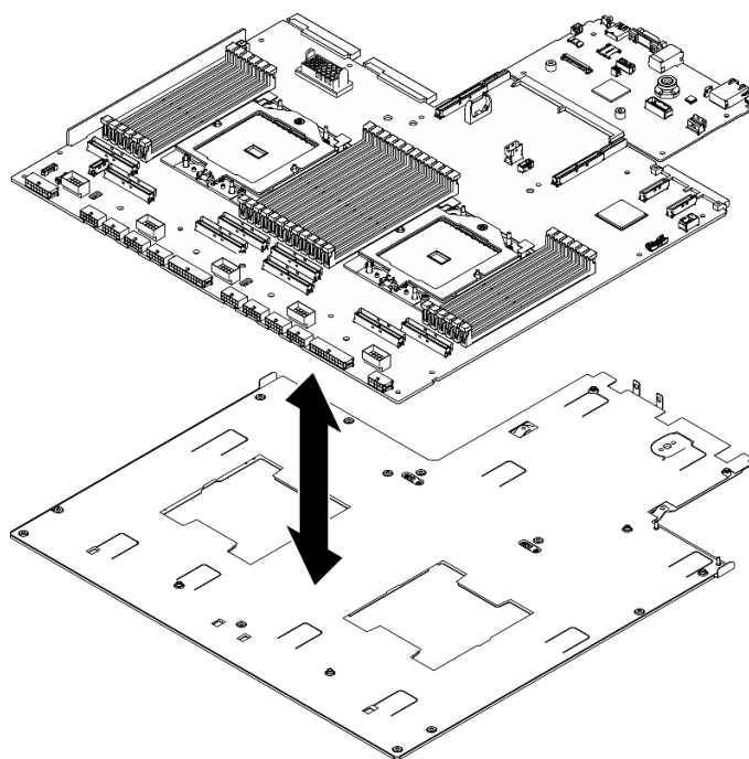
Figura 210. Instalação do conjunto de placa-mãe
