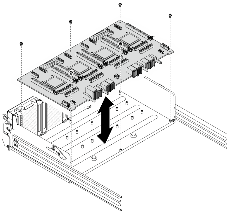
Figura 143. Remoção do Placa de comutador PCIe
