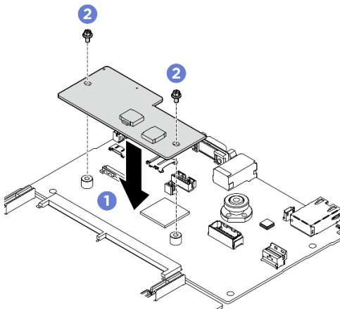
Figura 199. Instalação do Firmware e o módulo de segurança RoT
