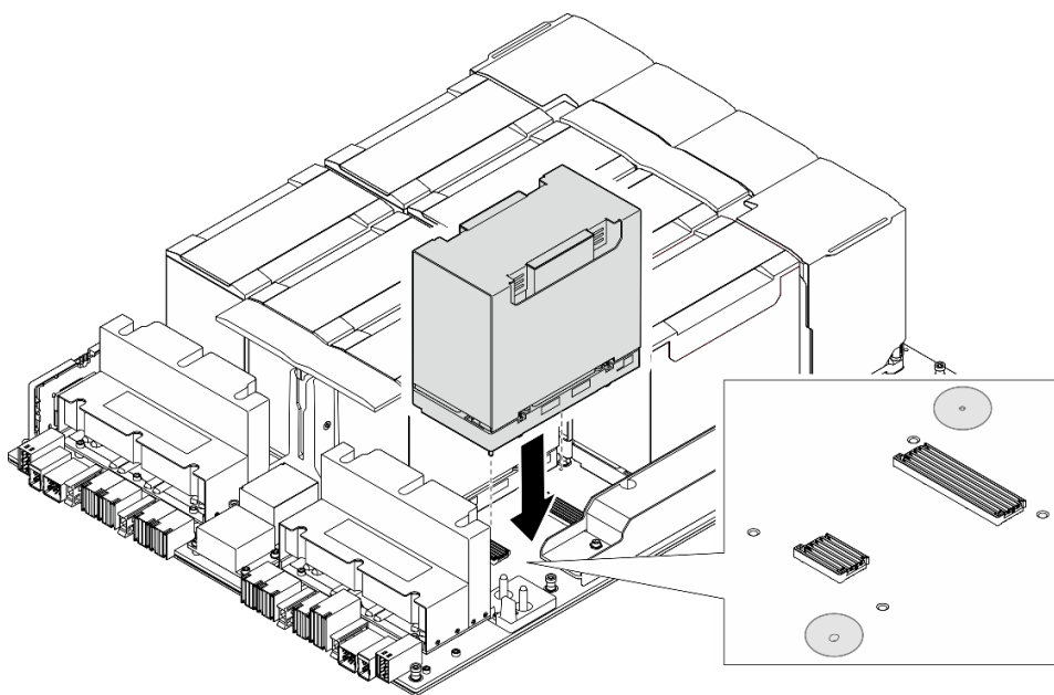
Figura 98. Instalação do Módulo de GPU e dissipador de calor
