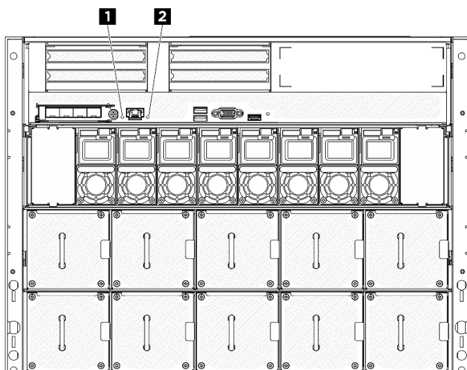
Figura 252. LEDs do sistema na vista traseira
