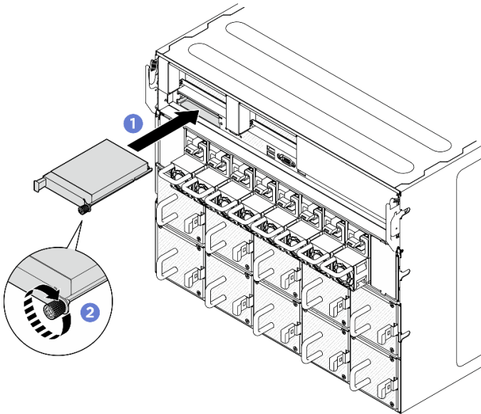
Figura 125. Instalação do módulo OCP
