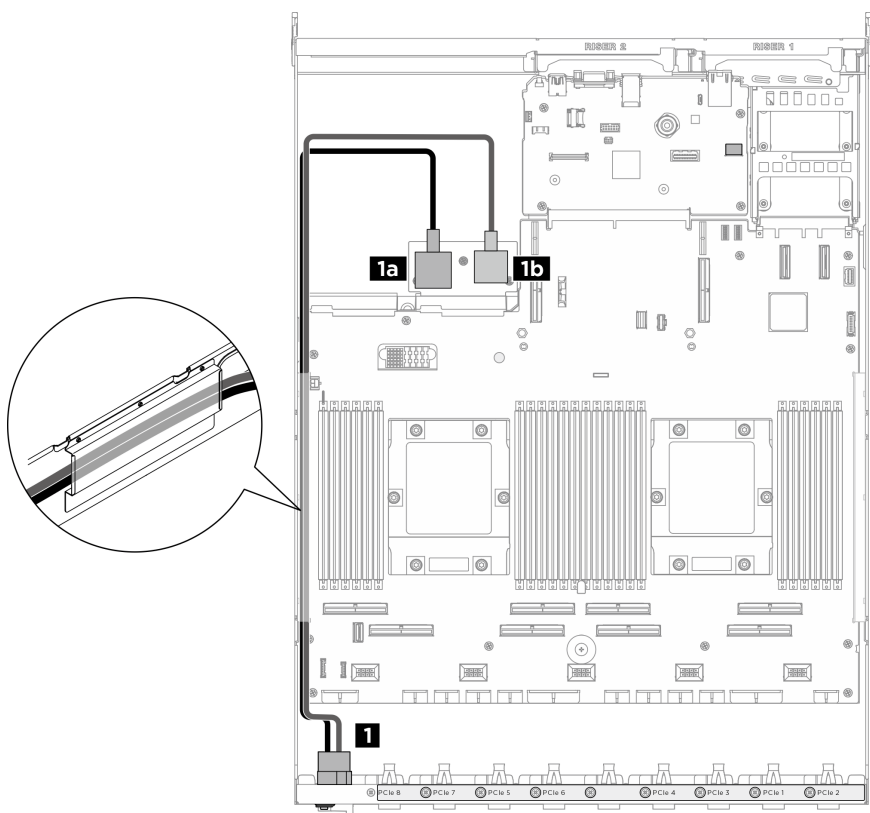
Figura 244. Roteamento de cabos da Placa de interface de alimentação
