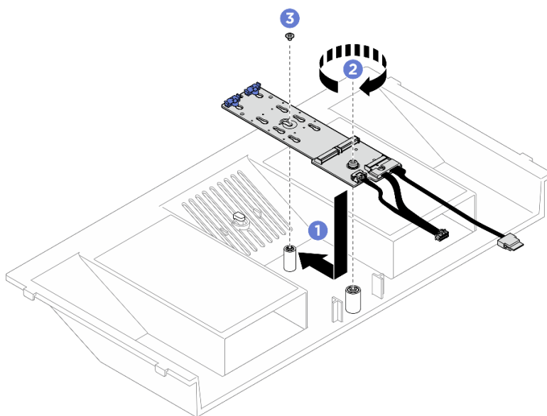
Figura 113. Instalação do backplane M.2
