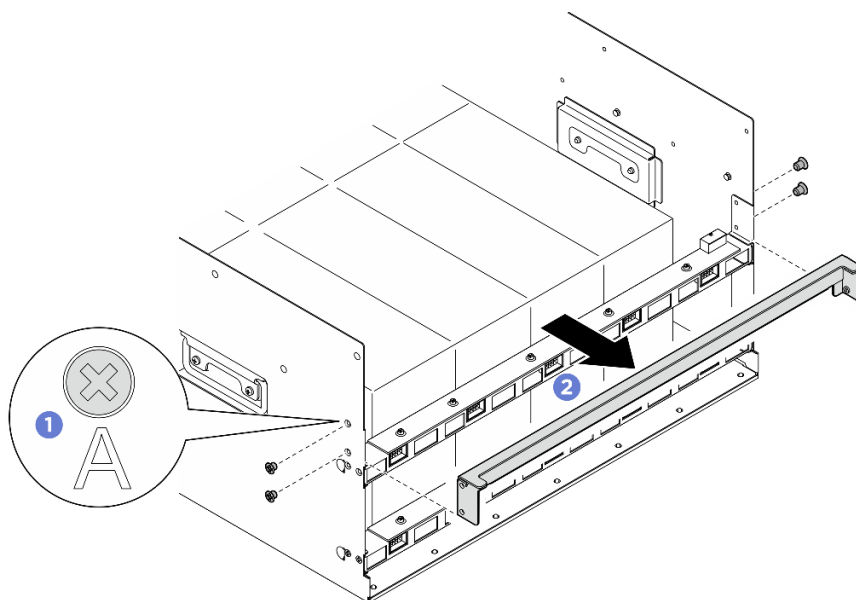
Figura 79. Remoção do suporte de apoio traseiro
