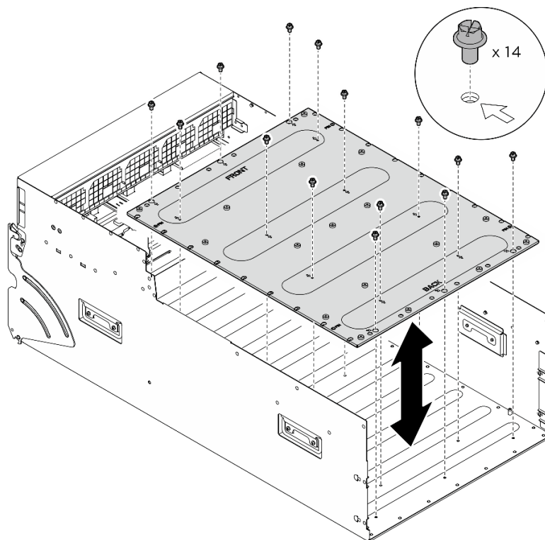
Figura 91. Remoção do Placa adaptadora do complexo da GPU
