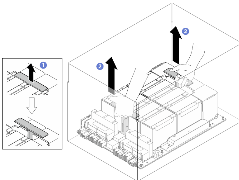
Figura 73. Removendo a Complexo da GPU da caixa de pacote
