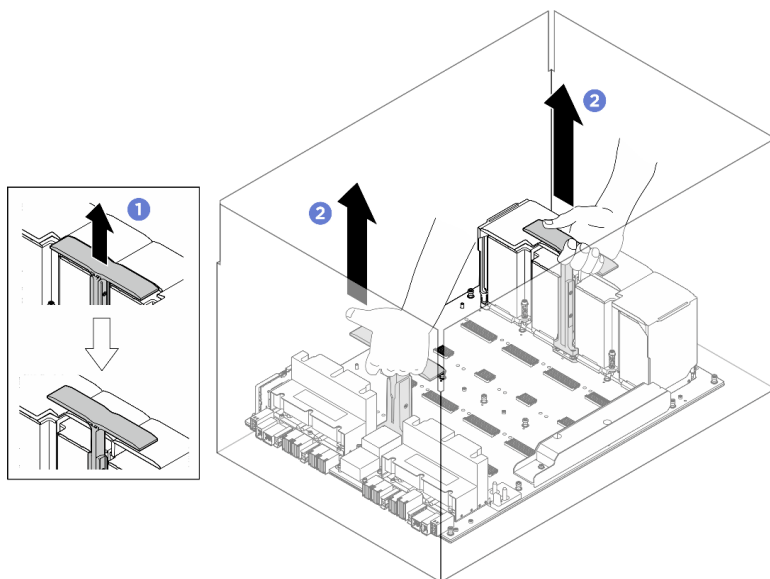
Figura 62. Removendo a Placa-base da GPU da caixa de pacote
