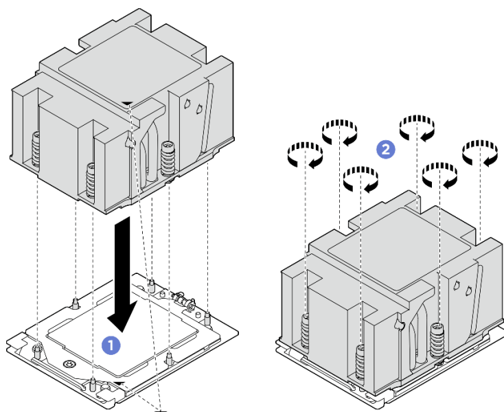
Figura 188. Instalação do dissipador de calor
