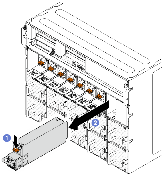
Figura 177. Remoção da unidade de fonte de alimentação
