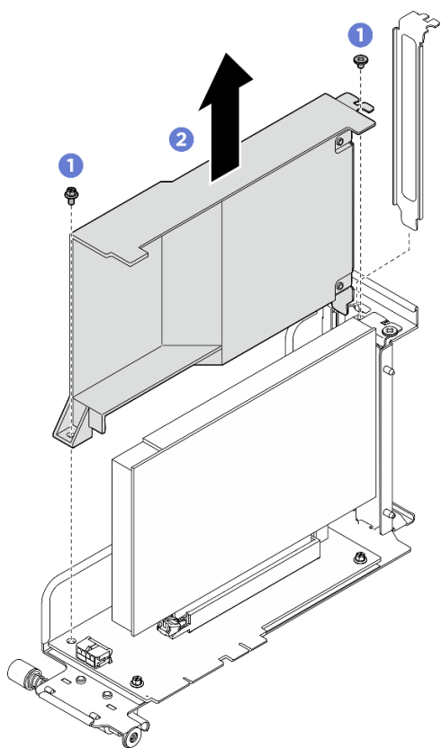
Figura 136. Remoção do defletor de ar da placa riser PCIe
