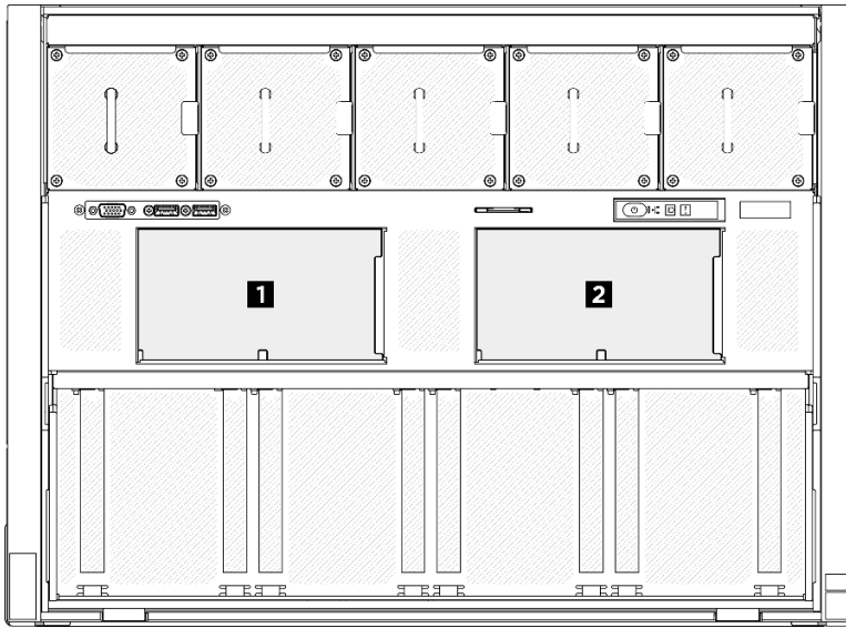
Figura 21. Numeração do backplane de unidade de 2,5 polegadas
