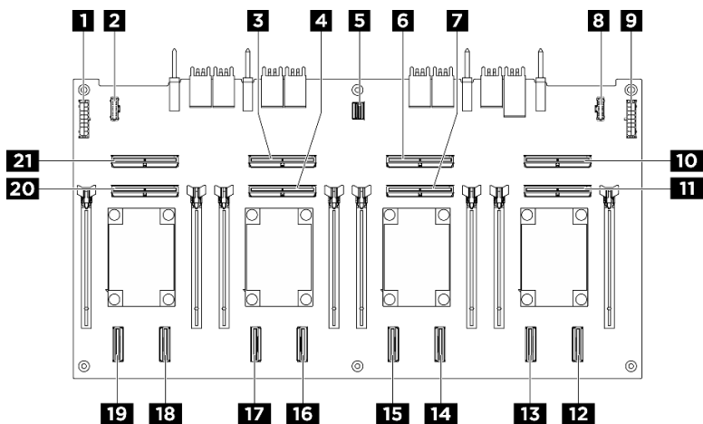
Figura 222. Conectores Placa de comutador PCIe
