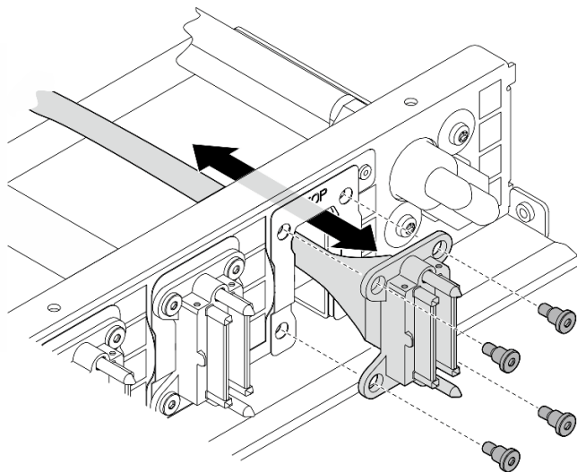
Figura 150. Remoção do módulo de E/S frontal, do painel de diagnóstico integrado, do gerenciamento de GPU ou do cabo de sinal
