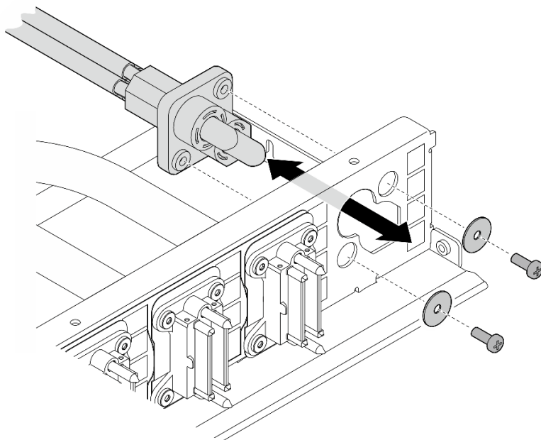
Figura 154. Instalação do cabo de alimentação
