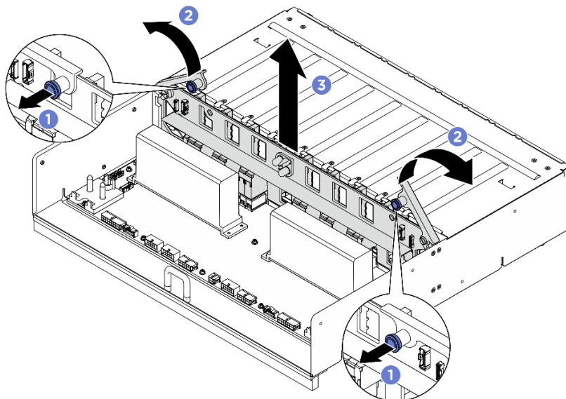
Figura 189. Remoção do Placa de interposição de PSU
