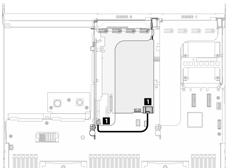
Figura 232. Roteamento de cabos do adaptador DPU
