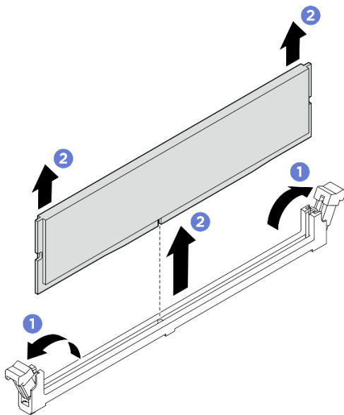
Figura 119. Remoção do módulo de memória
