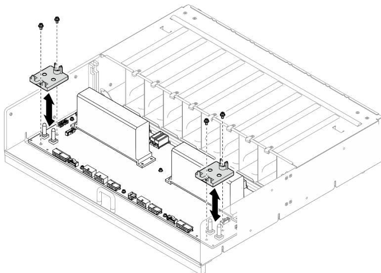
Figura 173. Instalação do retentor de cabos
