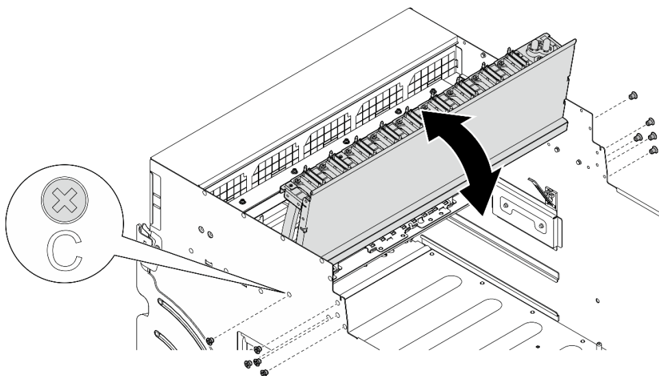
Figura 81. Virando o conjunto de cabos do comutador PCIe frontal
