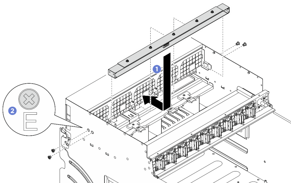
Figura 43. Instalação do conjunto de placa de controle do ventilador frontal
