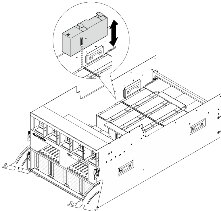
Figura 53. Remoção do duto de ar da GPU
