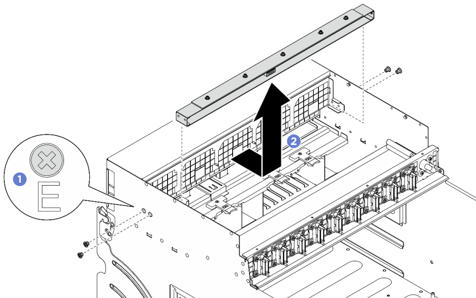
Figura 40. Remoção do conjunto de placa de controle do ventilador frontal
