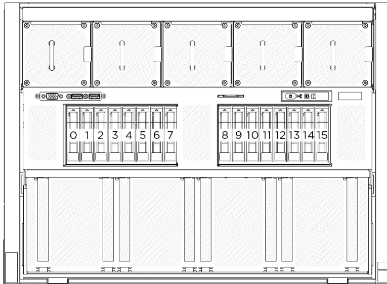
Figura 17. Numeração do compartimento de unidade de 2,5 polegadas
