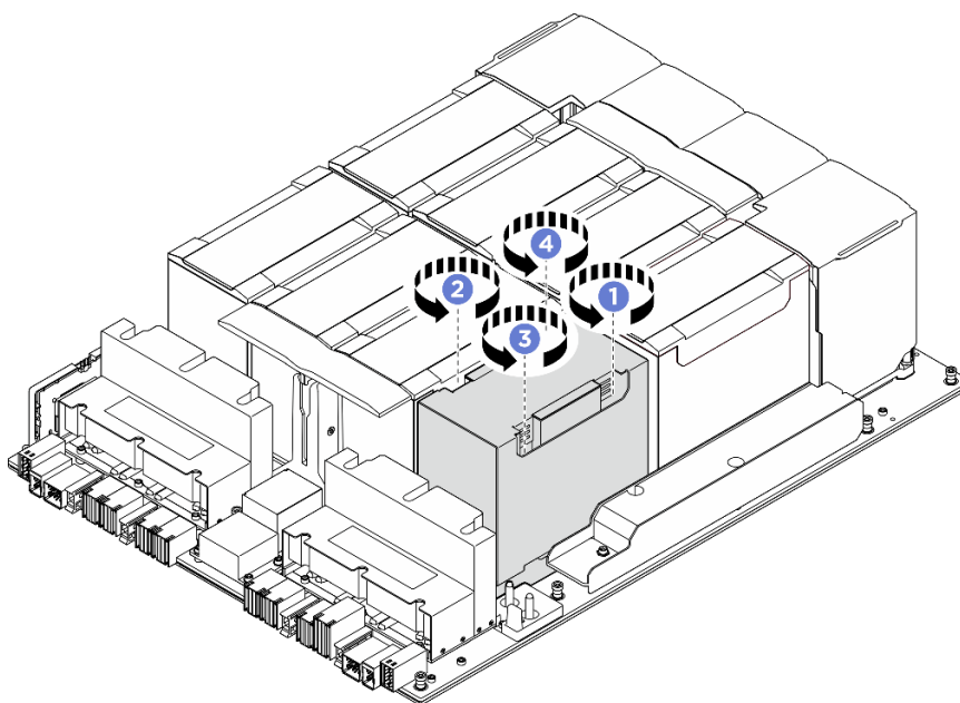
Figura 99. Sequência de aperto dos parafusos
