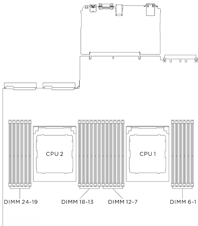
Figura 118. Layout de módulos de memória e processadores
