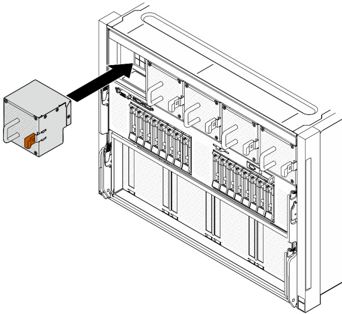
Figura 39. Instalação do ventilador hot-swap
