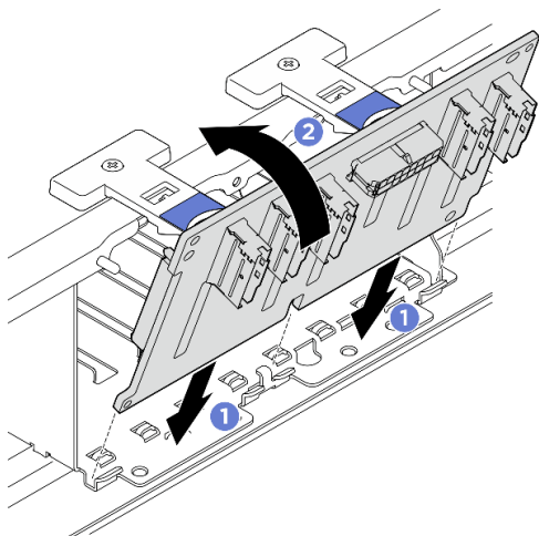
Figura 24. Instalação do painel traseiro da unidade de 2,5 polegadas
