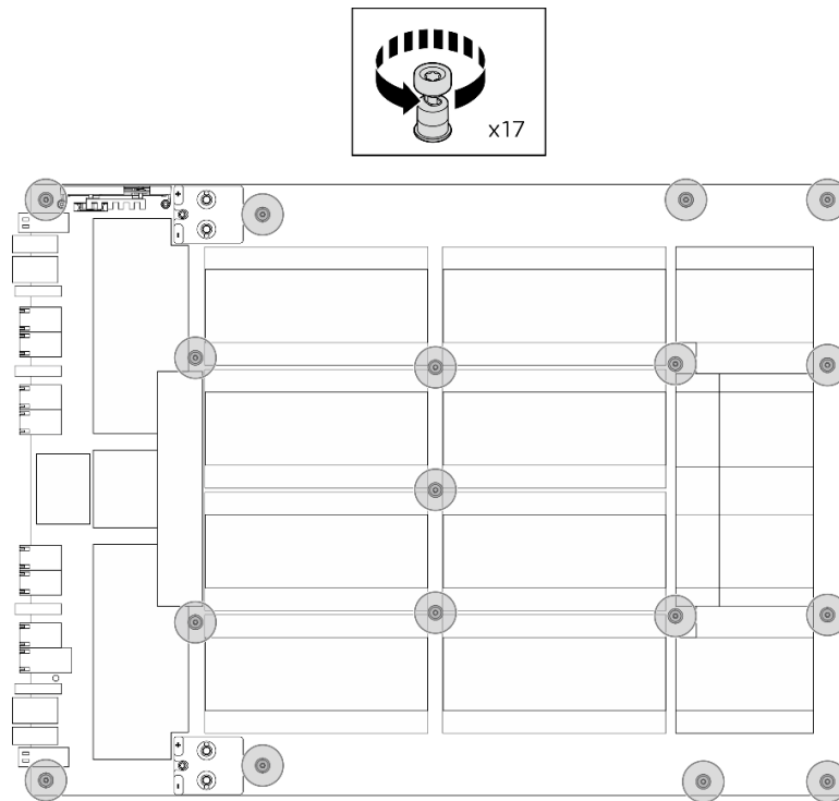
Figura 60. Remoção do parafuso
