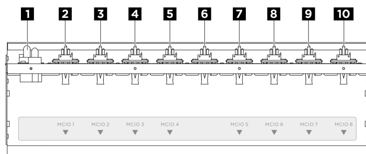
Figura 223. Cabos do conjunto de cabos do comutador PCIe frontal
