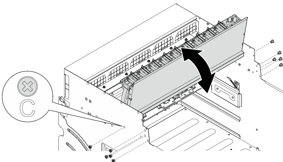
Figura 76. Virando o conjunto de cabos do comutador PCIe frontal
