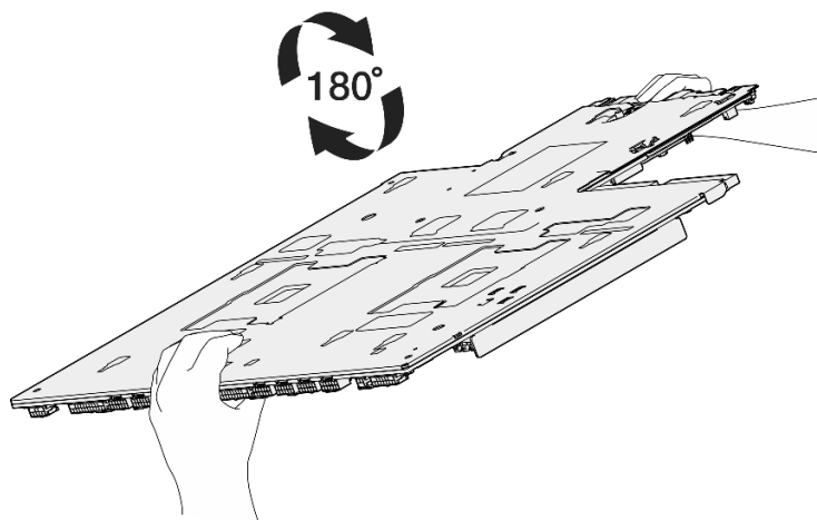
Figura 205. Girando o conjunto de placa-mãe lado direito para cima
