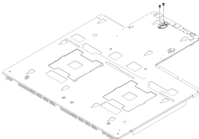
Figura 204. Remoção do parafuso
