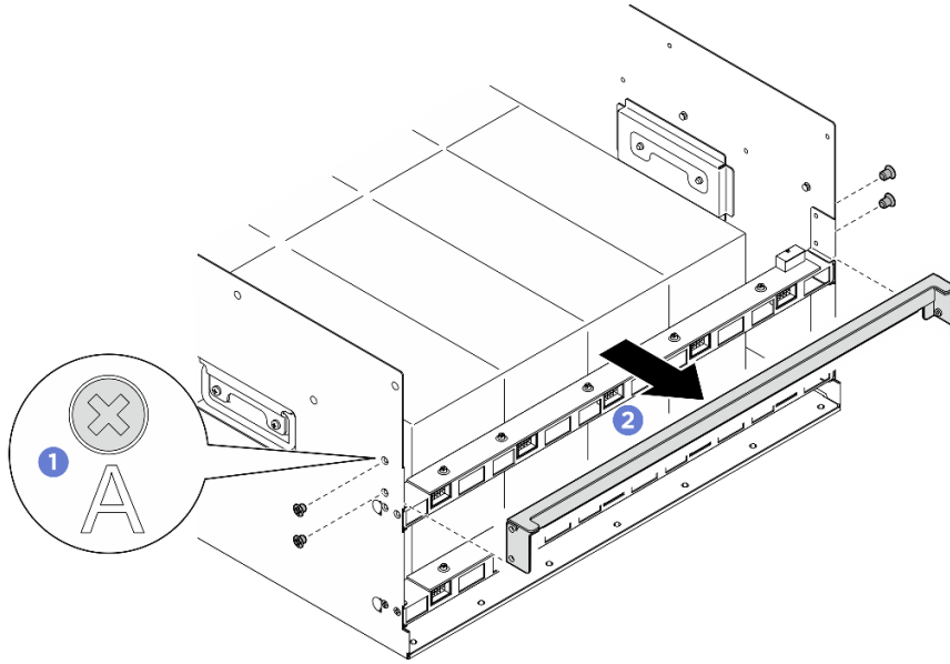
Figura 57. Remoção do suporte de apoio traseiro
