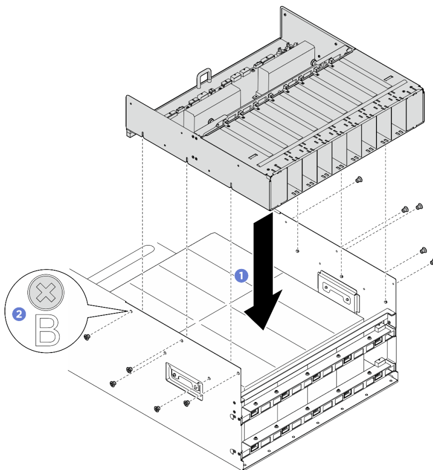
Figura 169. Instalação do Complexo de energia
