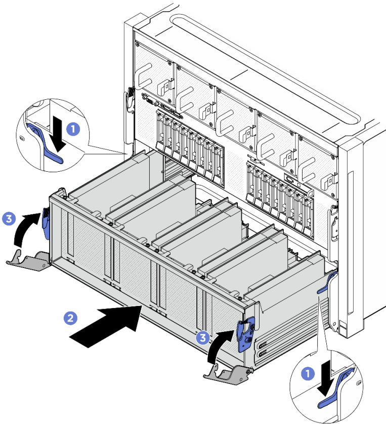
Figura 77. Instalação do Alternador do comutador PCIe no Alternador de GPU 8U
