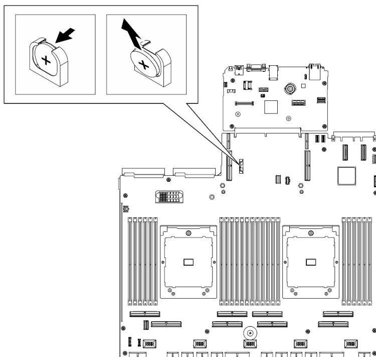
Figura 32. Remoção da bateria CMOS
