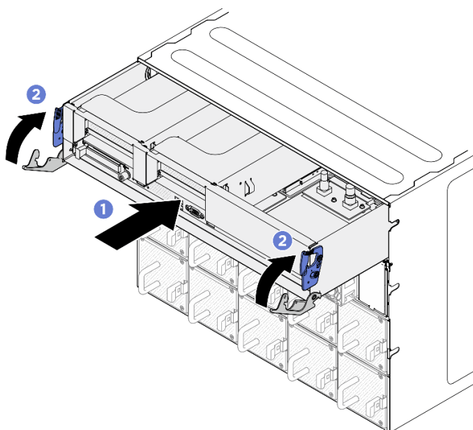
Figura 27. Instalação do Alternador de cálculo 2U
