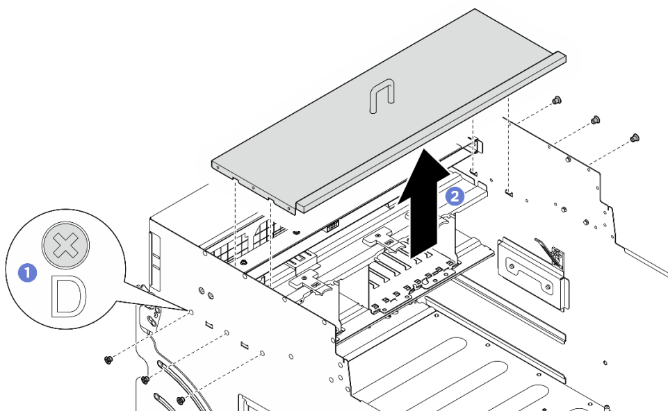
Figura 107. Remoção da tampa de E/S
