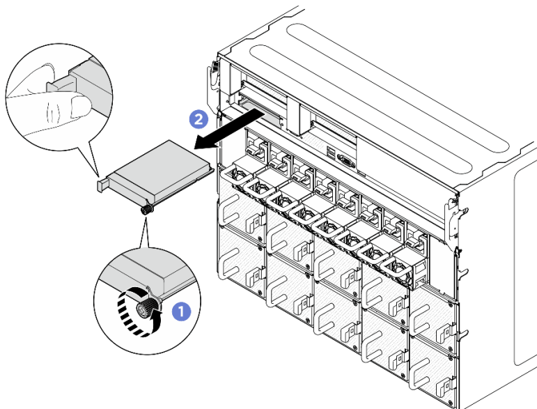
Figura 124. Remoção do módulo OCP
