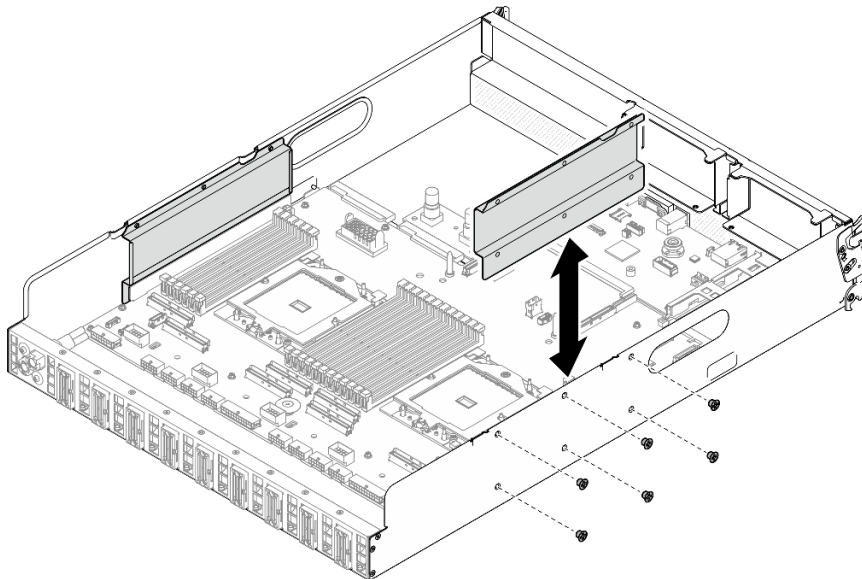
Figura 200. Remoção do guia de cabos
