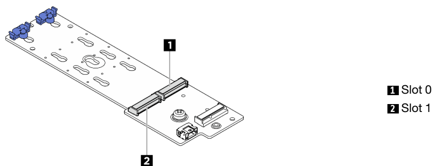
Figura 116. Slot da unidade M.2
