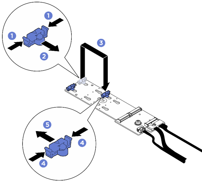
Figura 115. Ajuste do retentor do backplane M.2
