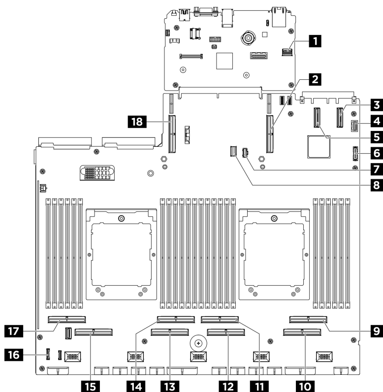
Figura 228. Conectores do conjunto da placa-mãe para roteamento de cabos
