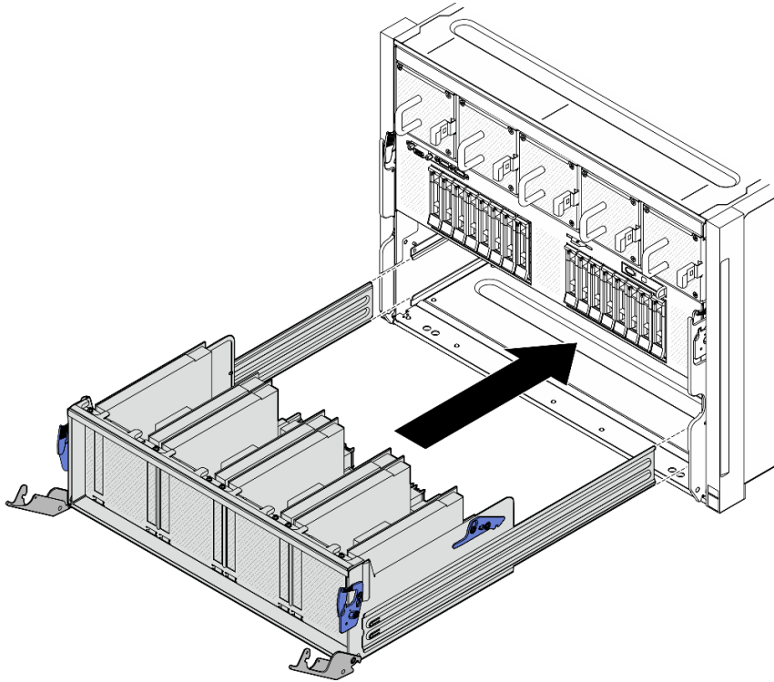
Figura 166. Instalação do Alternador do comutador PCIe na posição de parada
