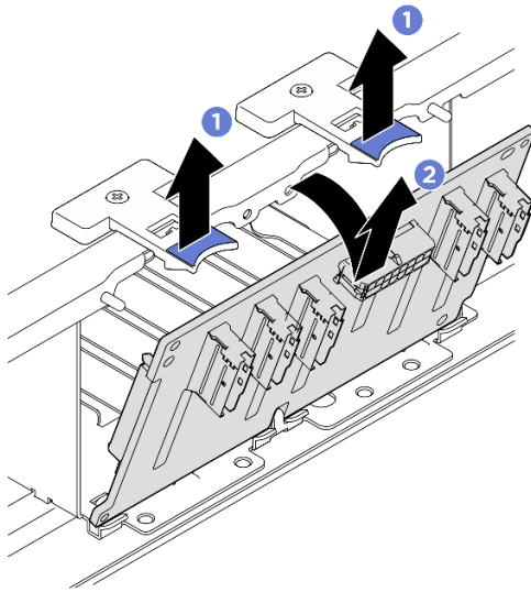
Figura 22. Remoção do painel traseiro da unidade de 2,5 polegadas
