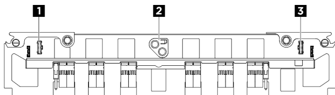
Figura 227. Conectores Placa de interposição de PSU
