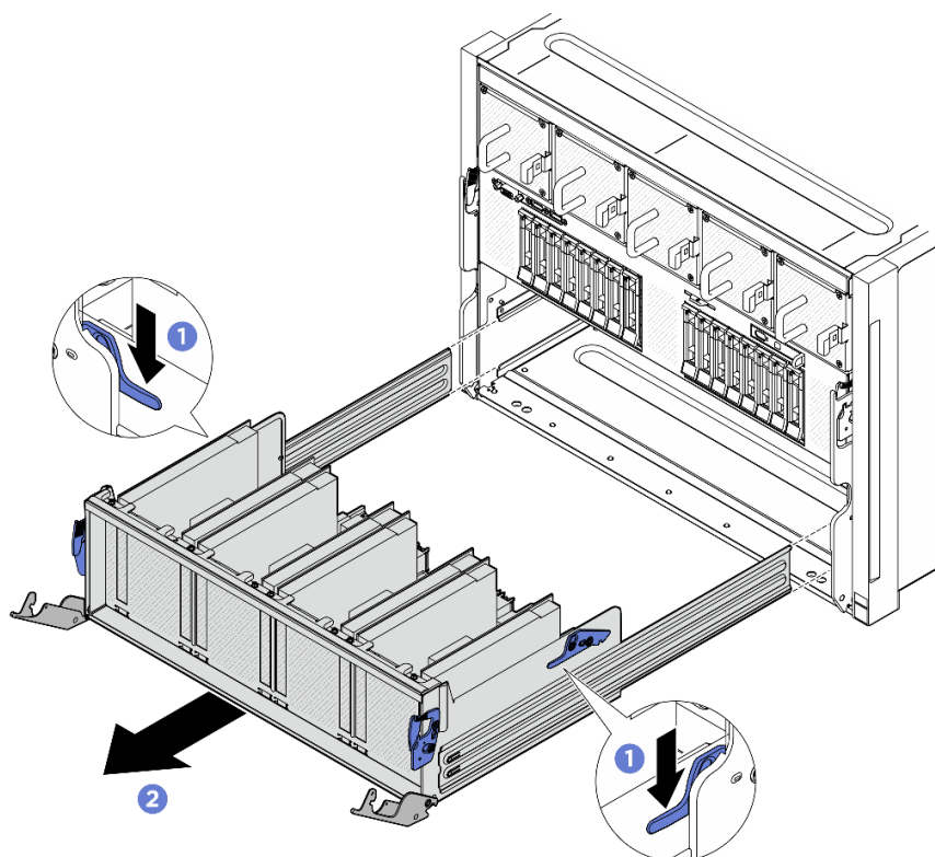
Figura 165. Alternador do comutador PCIe remoção do Alternador de GPU 8U
