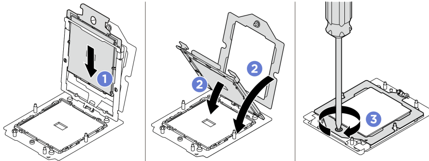
Figura 186. Instalação do processador
