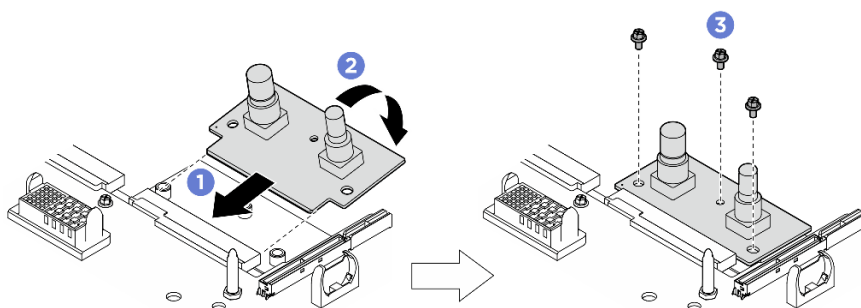
Figura 175. Instalação da placa de interface de alimentação
