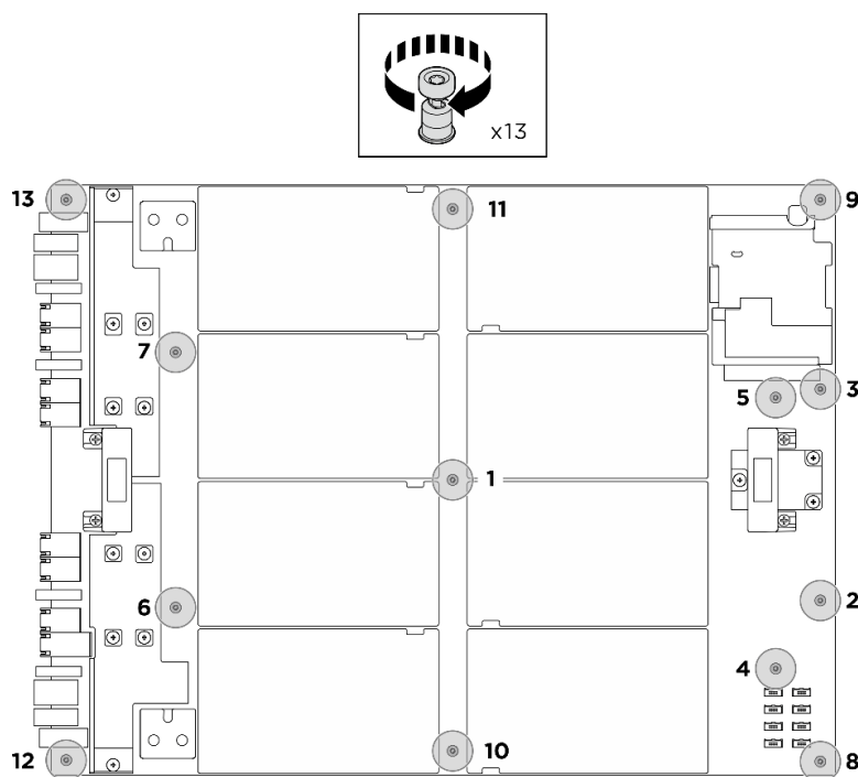
Figura 85. Instalação do parafuso
