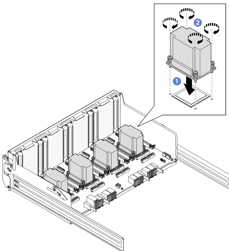
Figura 146. Instalação do Dissipador de calor da placa de comutador PCIe
