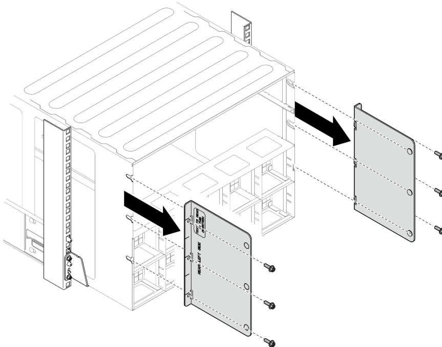
Figura 2. Remoção do suporte de apoio superior
