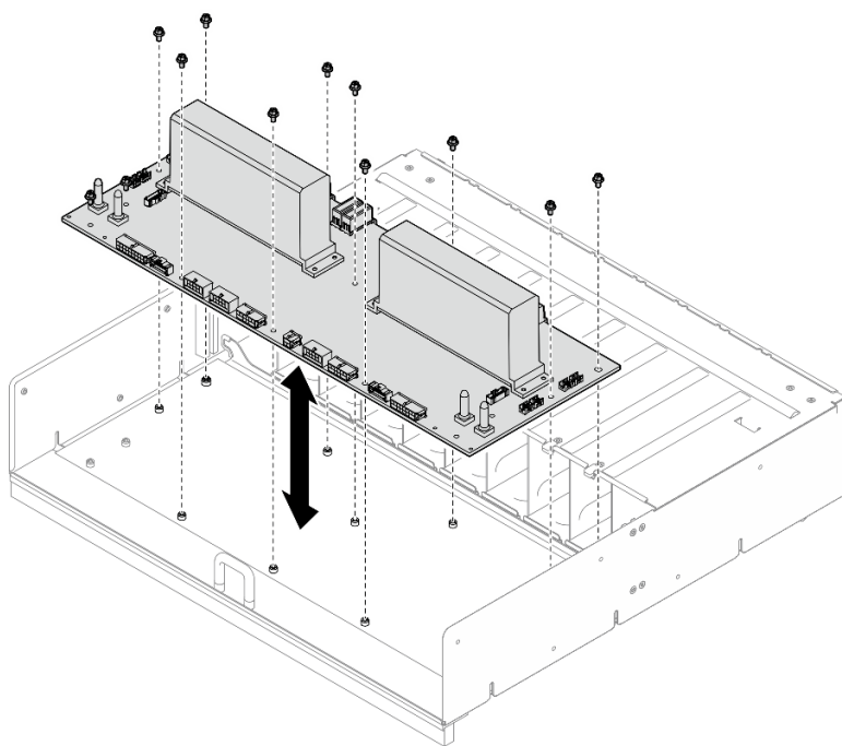
Figura 192. Instalação da placa de distribuição de energia
