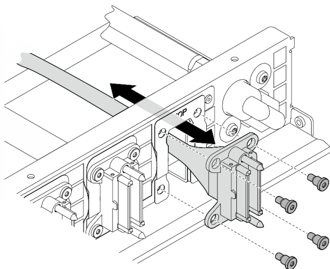
Figura 153. Módulo de E/S frontal, painel integrado de diagnósticos, gerenciamento de GPU ou instalação de cabo de sinal
