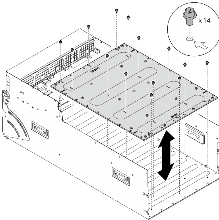
Figura 92. Instalação do Placa adaptadora do complexo da GPU
