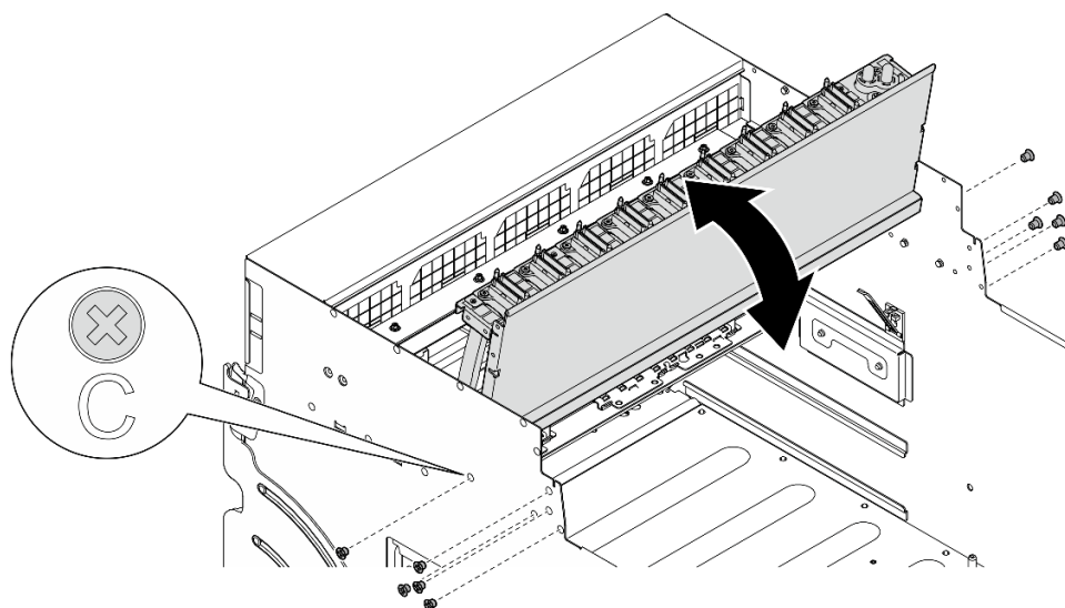
Figura 65. Virando o conjunto de cabos do comutador PCIe frontal
