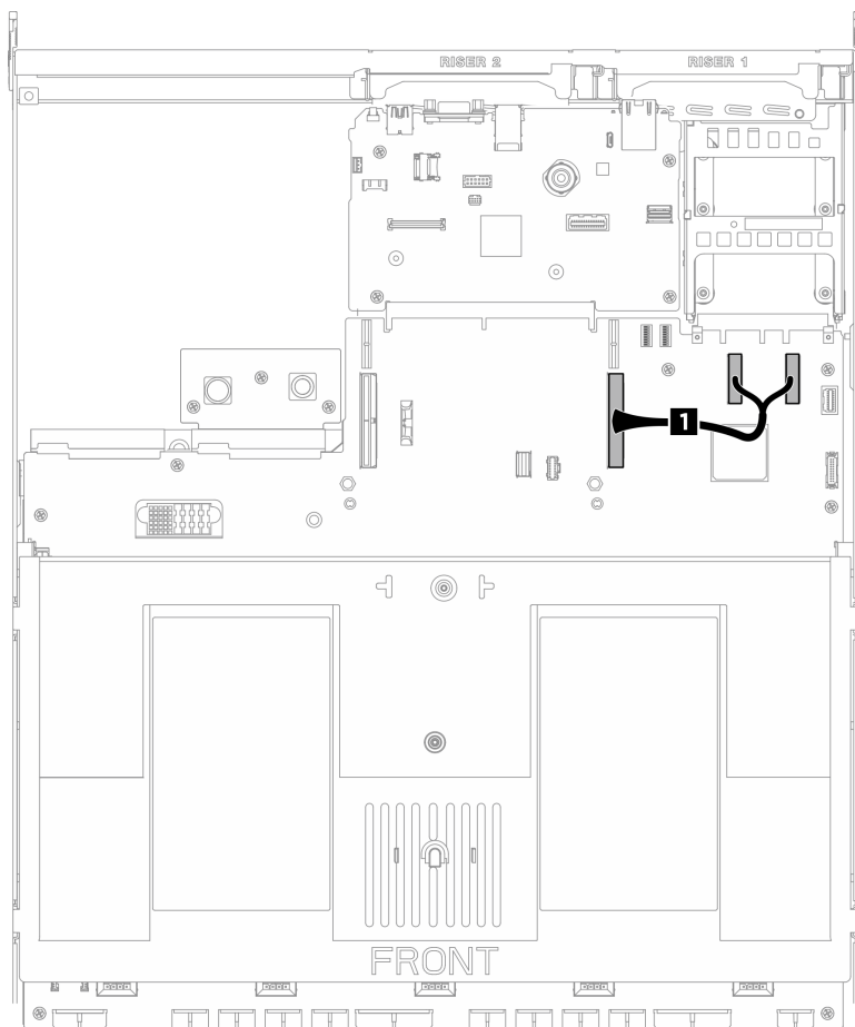
Figura 239. Roteamento de cabos do módulo OCP
