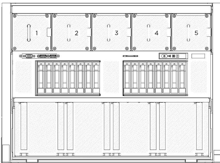
Figura 37. Numeração do ventilador frontal
