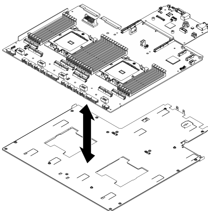
Figura 207. Desmontagem do conjunto da placa-mãe
