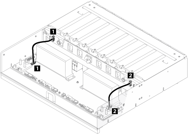
Figura 246. Roteamento de cabos da Placa de interposição de PSU
