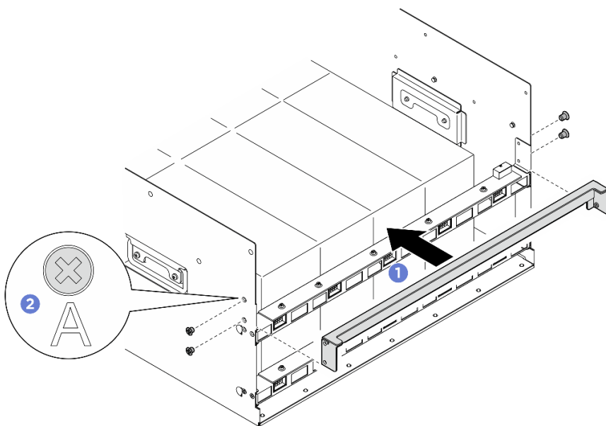
Figura 78. Instalação do suporte de apoio traseiro
