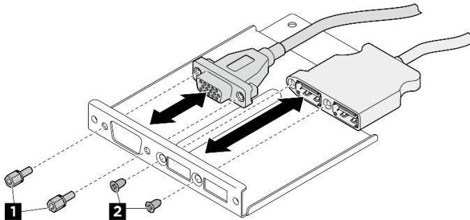
Figura 156. Instalação dos cabos do módulo de E/S frontal
