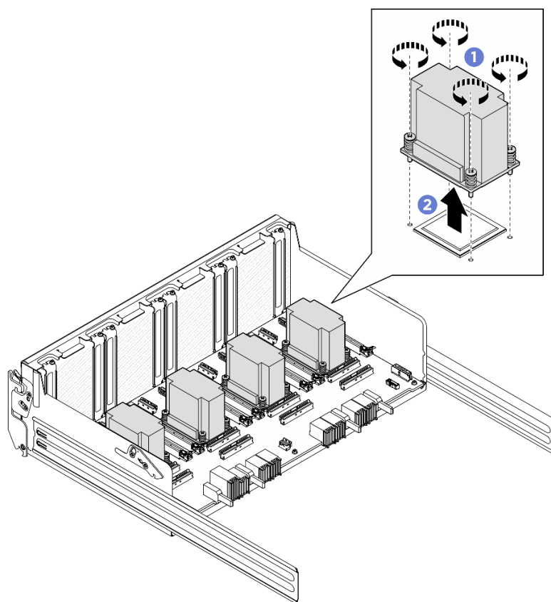
Figura 142. Remoção do Dissipador de calor da placa de comutador PCIe
