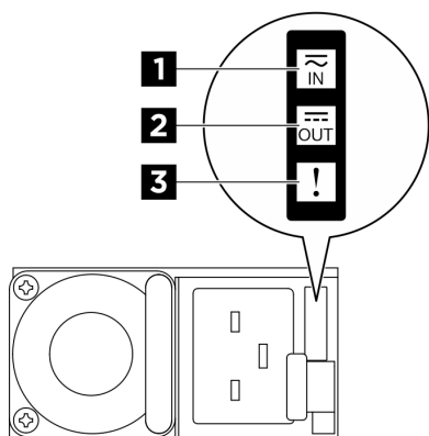
Figura 251. LEDs da fonte de alimentação CFFv4
