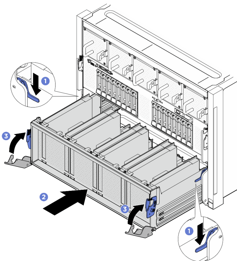
Figura 94. Instalação do Alternador do comutador PCIe no Alternador de GPU 8U
