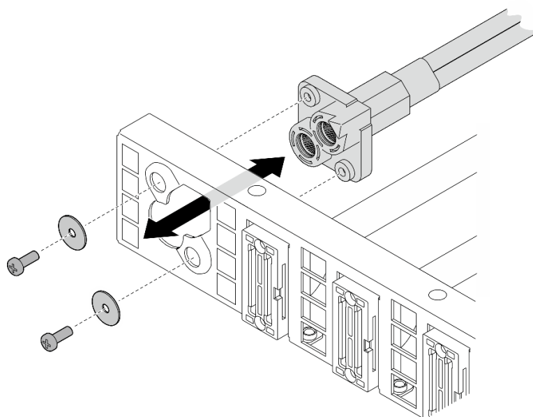
Figura 160. Remoção do cabo de alimentação
