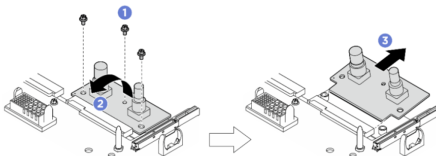
Figura 190. Remoção da placa de interface de energia
