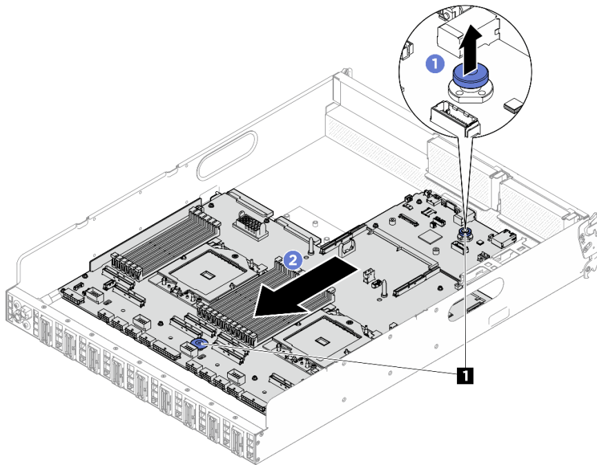
Figura 217. Desencaixe do conjunto da placa-mãe
