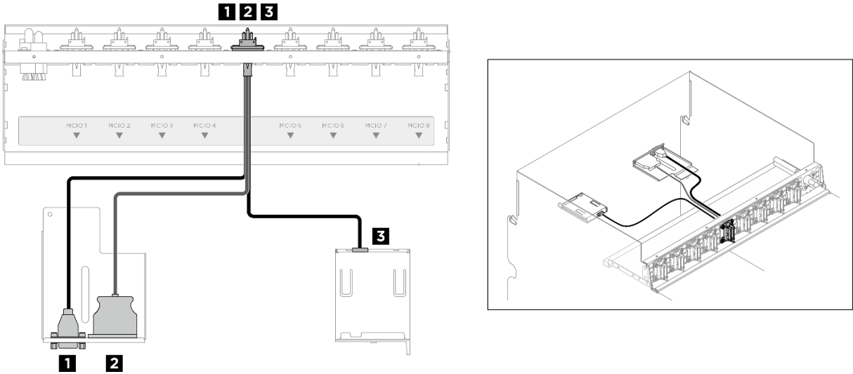
Figura 254. Roteamento de cabos do módulo de E/S frontal e do painel de diagnóstico integrado
