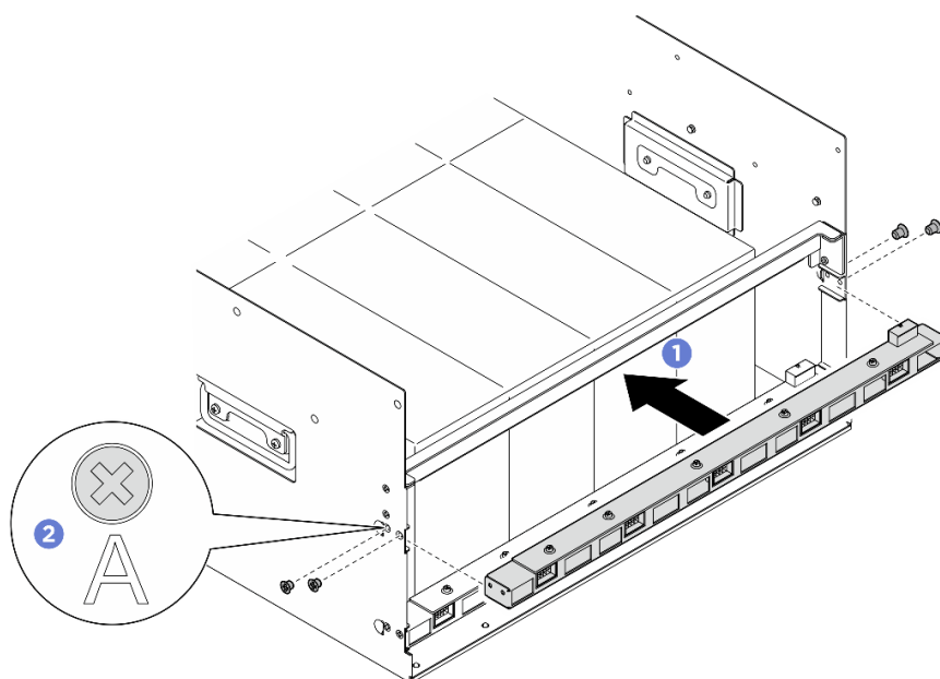
Figura 64. Instalação do conjunto placa de controle do ventilador traseiro
