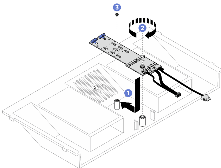
Figura 129. Instalação do backplane M.2
