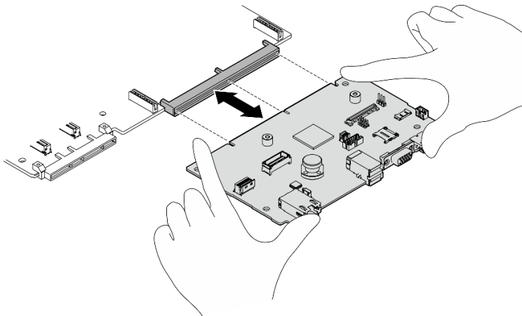
Figura 225. Instalação da placa de E/S do sistema
