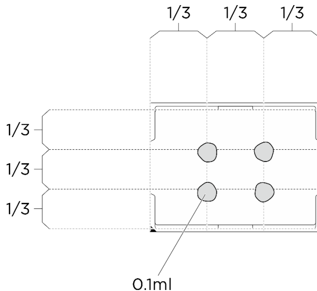
Figura 203. Aplicação de graxa térmica
