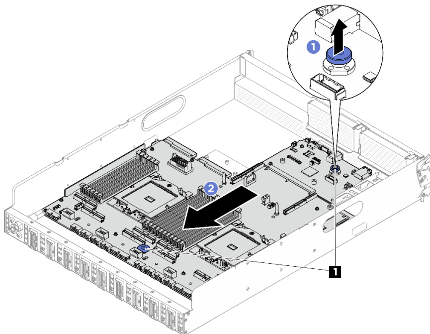
Figura 270. Desencaixe do conjunto da placa-mãe
