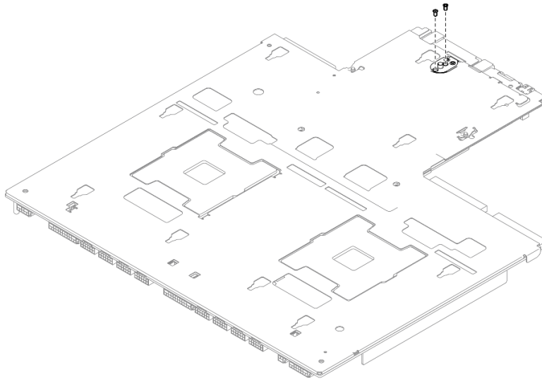
Figura 273. Remoção do parafuso
