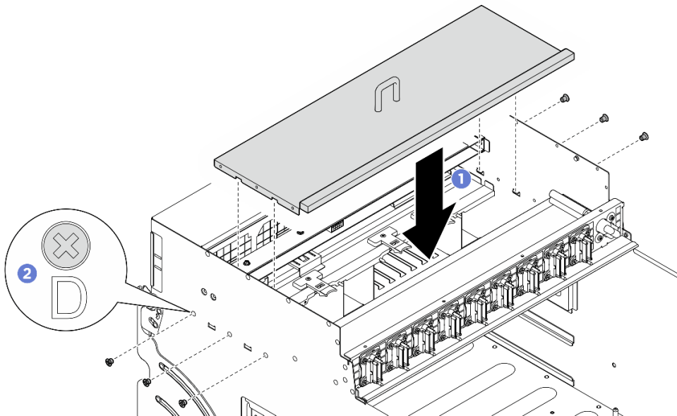
Figura 124. Instalação da tampa de E/S
