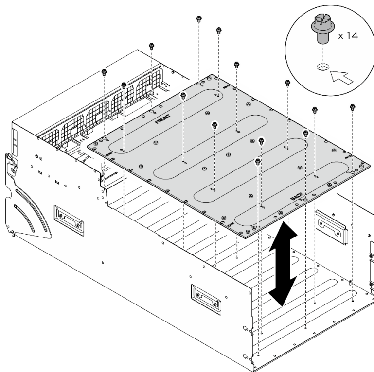
Figura 107. Remoção do Placa adaptadora do complexo da GPU
