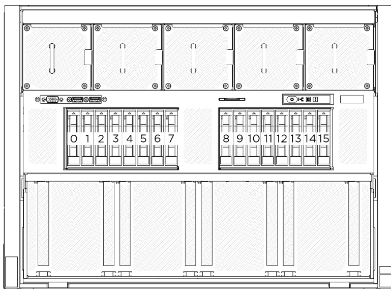
Figura 35. Numeração do compartimento de unidade de 2,5 polegadas
