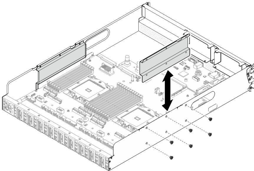
Figura 269. Remoção do guia de cabos
