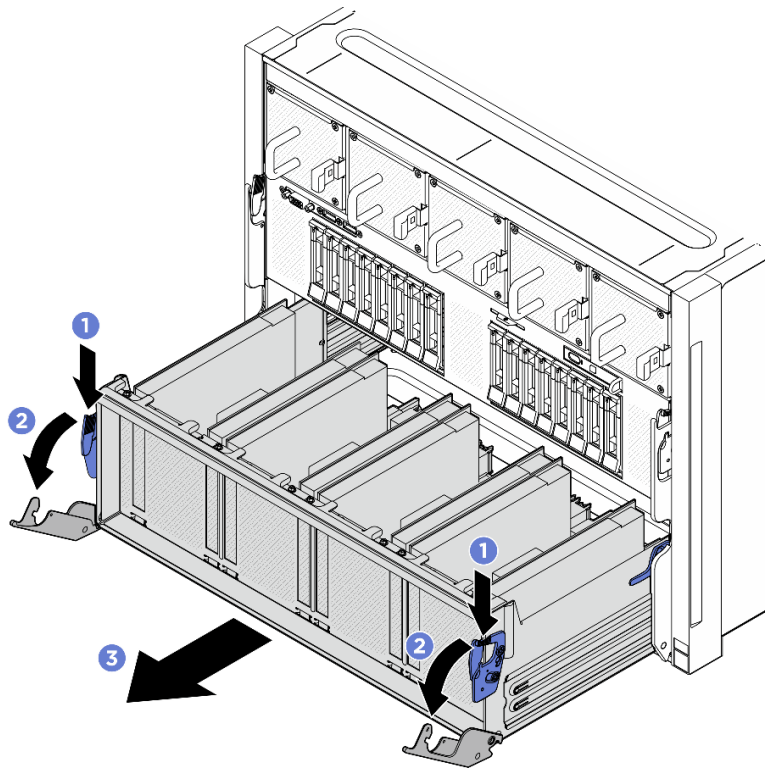
Figura 142. Remoção do Alternador do comutador PCIe para a posição de parada
