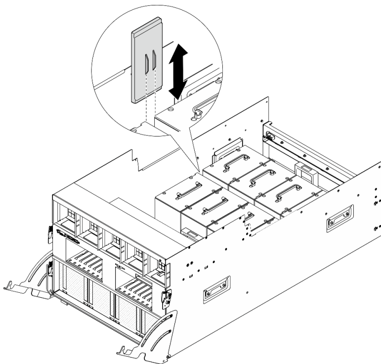
Figura 72. Instalação do duto de ar da GPU
