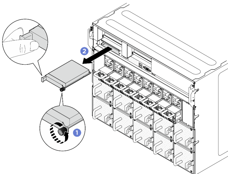
Figura 140. Remoção do módulo OCP
