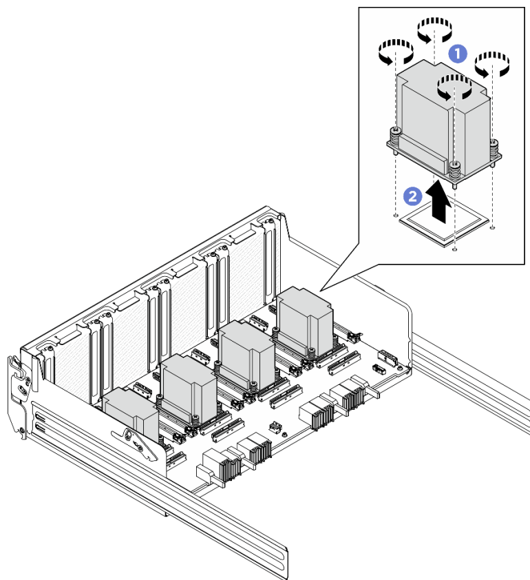
Figura 158. Remoção do Dissipador de calor da placa de comutador PCIe
