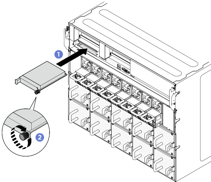
Figura 141. Instalação do módulo OCP
