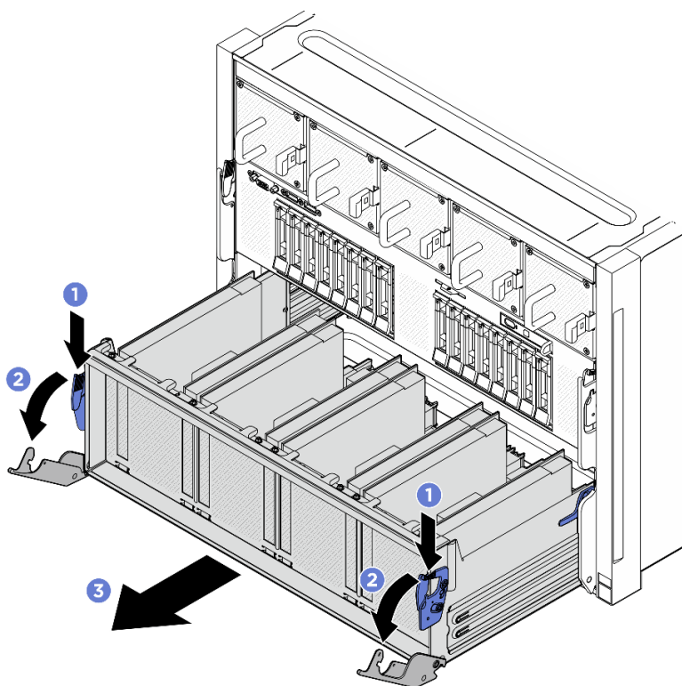
Figura 85. Remoção do Alternador do comutador PCIe para a posição de parada
