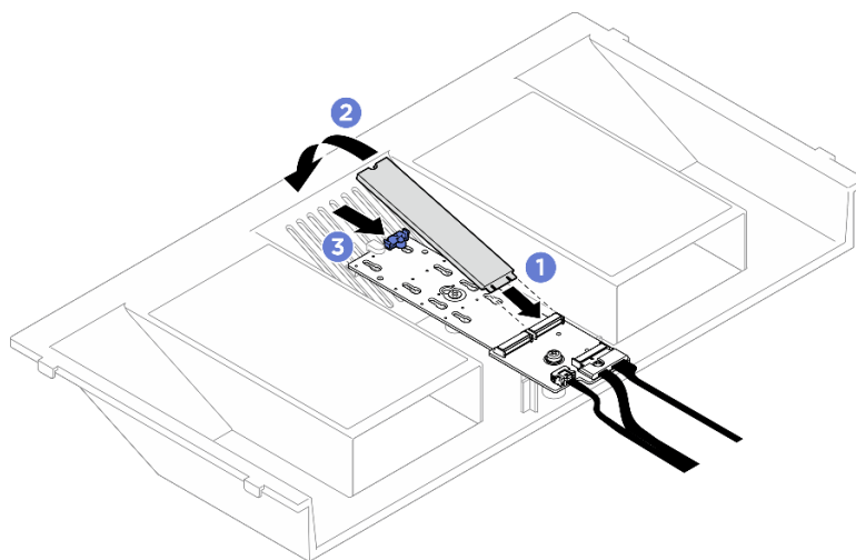
Figura 133. Instalação da unidade M.2
