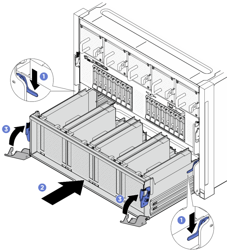
Figura 82. Instalação do Alternador do comutador PCIe no Alternador de GPU 8U
