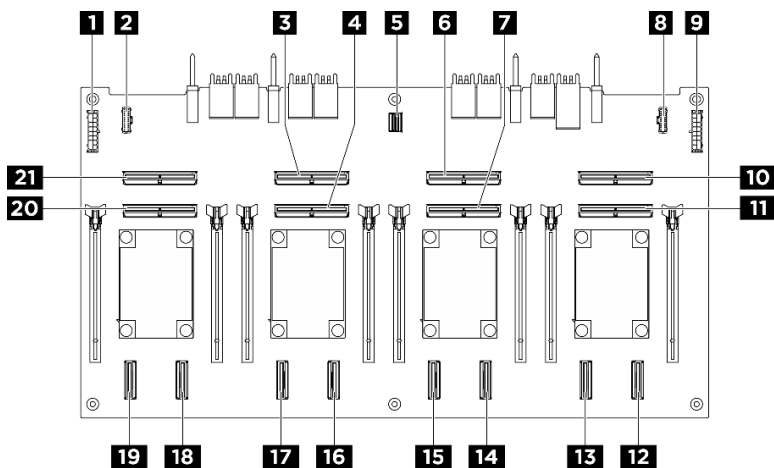
Figura 238. Conectores Placa de comutador PCIe
