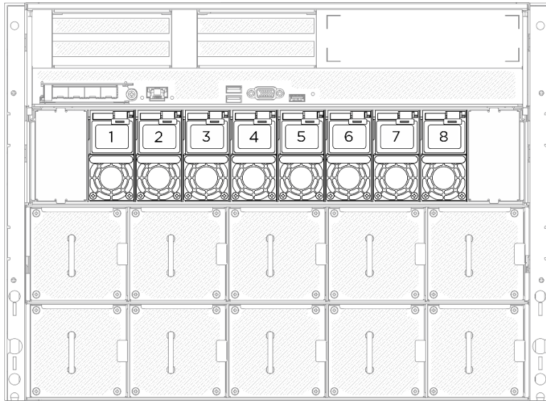
Figura 192. Numeração do preenchimento do compartimento de fonte de alimentação
