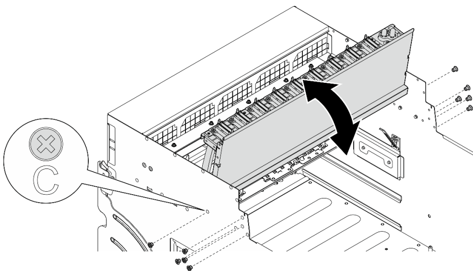
Figura 92. Virando o conjunto de cabos do comutador PCIe frontal
