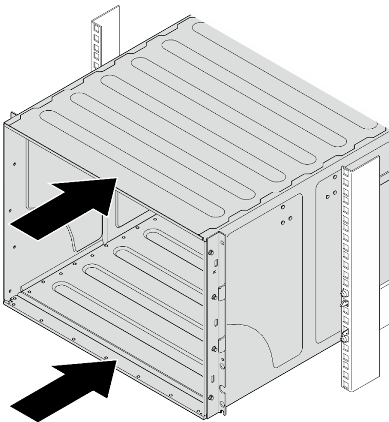
Figura 29. Deslizando o chassi
