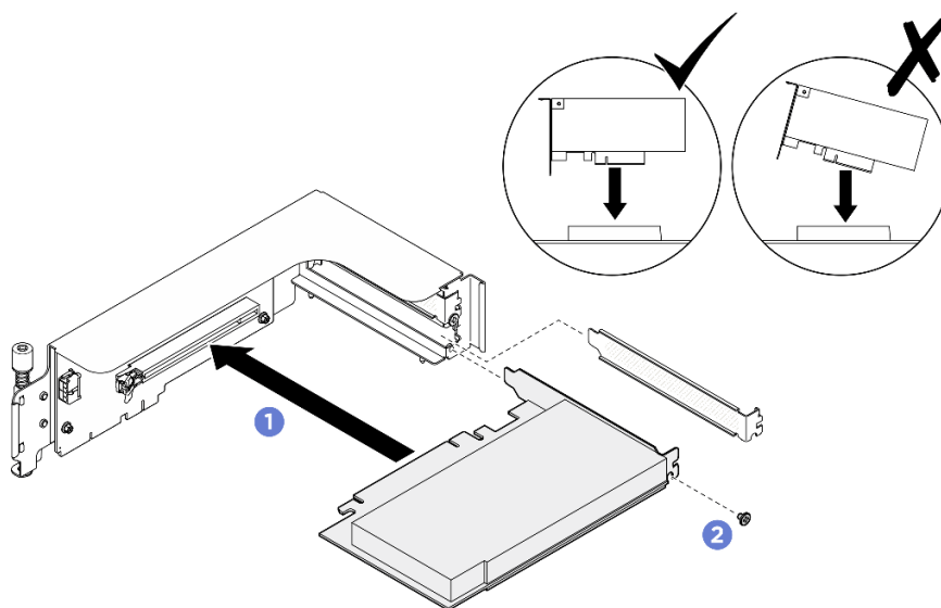
Figura 147. Instalação do adaptador PCIe traseiro
