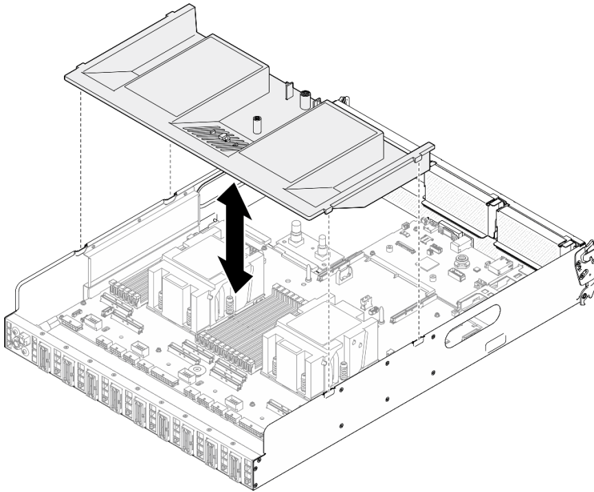
Figura 196. Remoção do defletor de ar do processador
