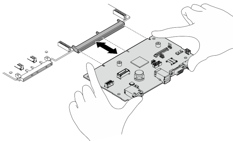
Figura 224. Remoção da placa de E/S do sistema
