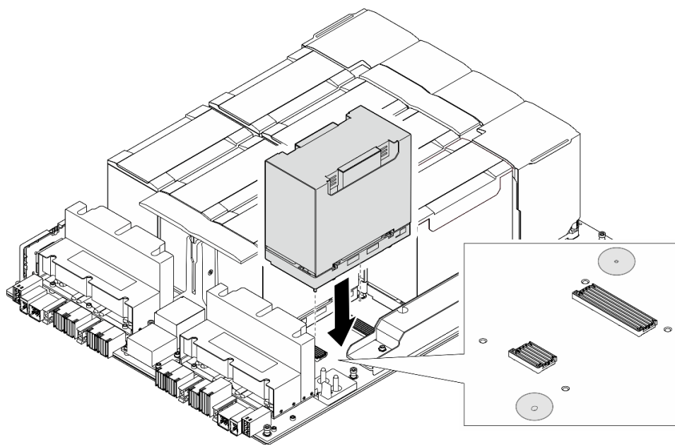
Figura 114. Instalação do Módulo de GPU e dissipador de calor
