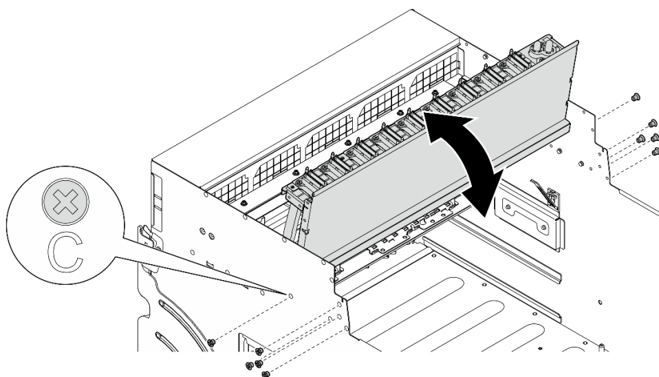
Figura 102. Virando o conjunto de cabos do comutador PCIe frontal
