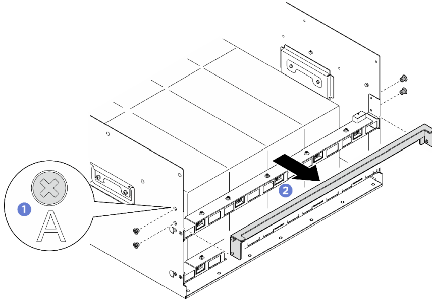
Figura 73. Remoção do suporte de apoio traseiro
