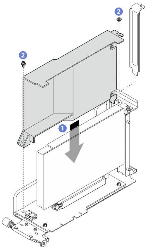
Figura 149. Instalação do defletor de ar da placa riser PCIe
