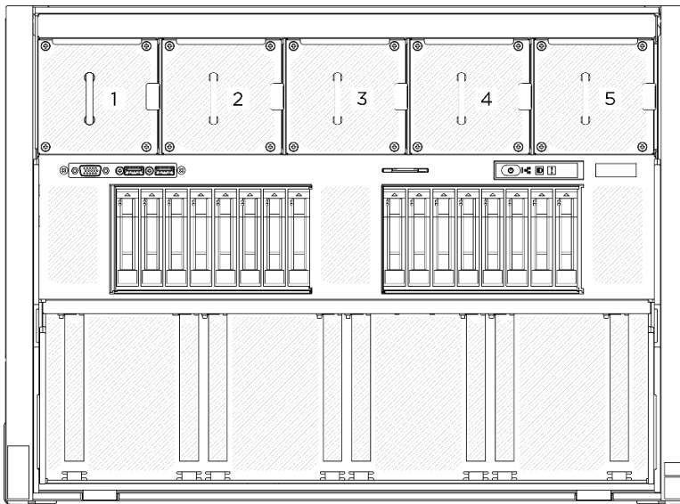
Figura 50. Numeração do ventilador frontal
