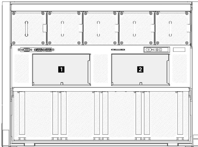
Figura 37. Numeração do backplane de unidade de 2,5 polegadas
