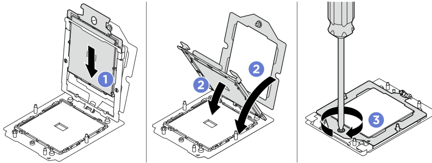
Figura 202. Instalação do processador
