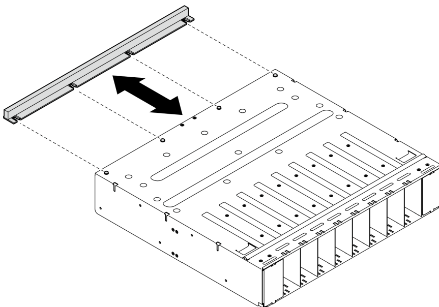
Figura 67. Remoção do defletor de ar da GPU
