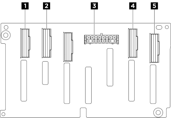
Figura 234. Conectores do backplane NVMe de 2,5 polegadas
