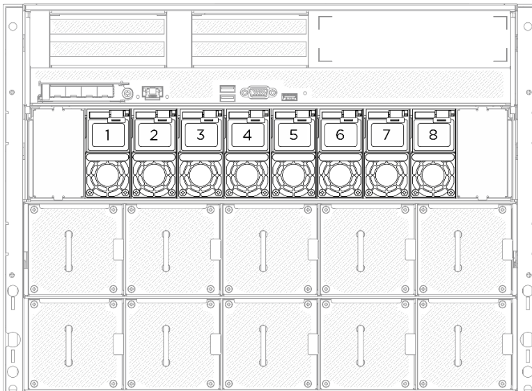
Figura 194. Numeração do preenchimento do compartimento de fonte de alimentação
