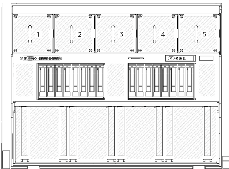
Figura 53. Numeração do ventilador frontal
