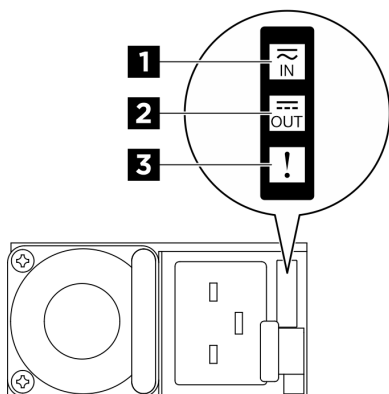
Figura 266. LEDs da fonte de alimentação CFFv4
