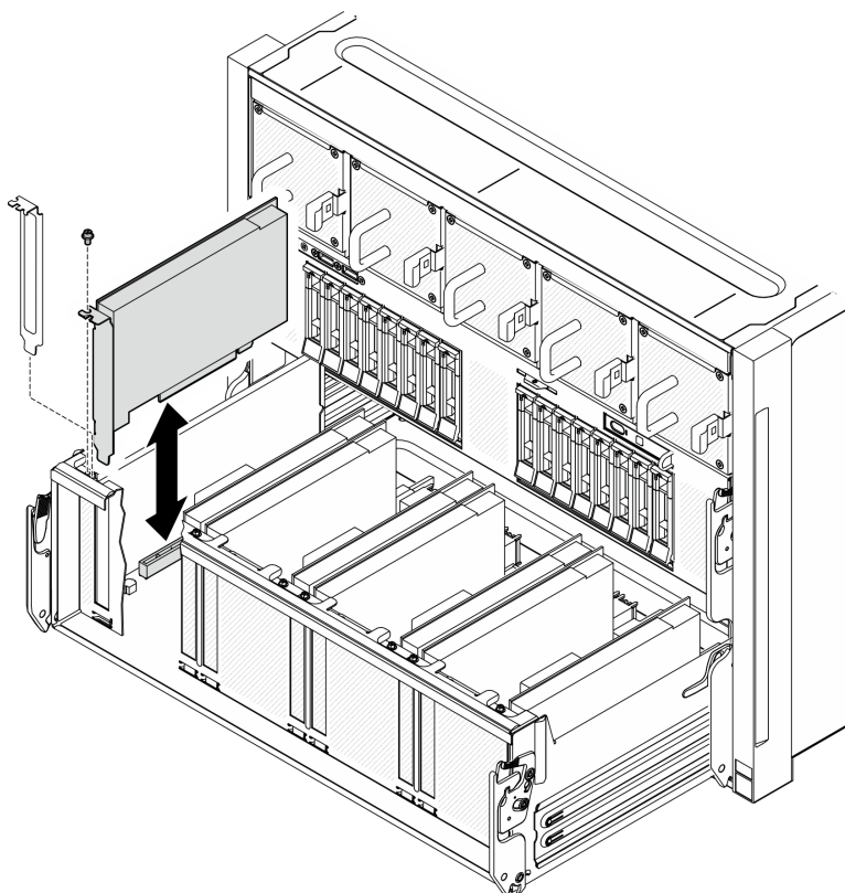
Figura 144. Instalação do adaptador PCIe frontal
