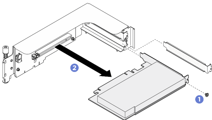
Figura 153. Remoção do adaptador PCIe traseiro
