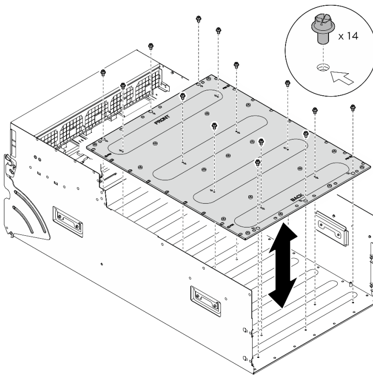
Figura 108. Instalação do Placa adaptadora do complexo da GPU
