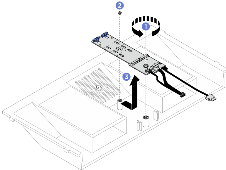
Figura 126. Remoção do backplane M.2
