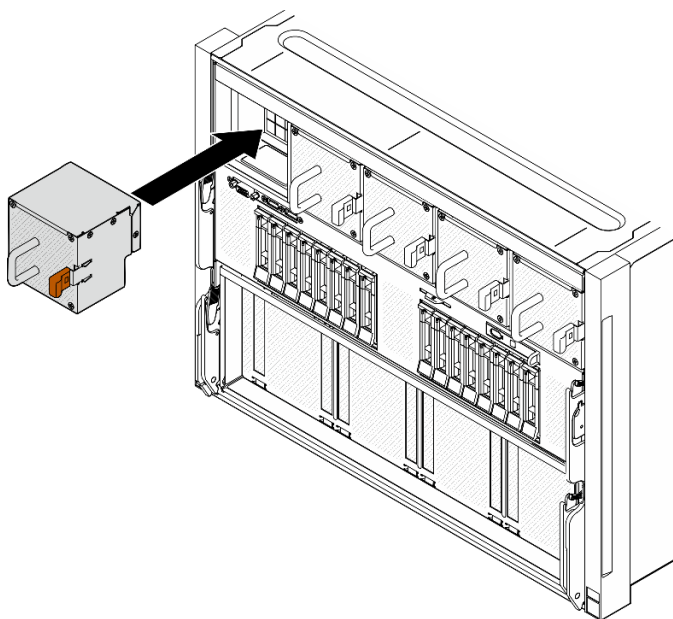
Figura 55. Instalação do ventilador hot-swap
