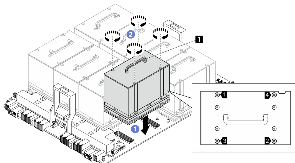
Figura 118. Instalação do Módulo de GPU e dissipador de calor
