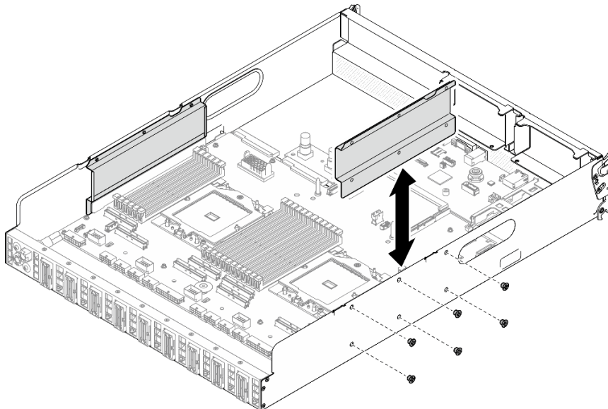
Figura 233. Instalação do guia de cabos
