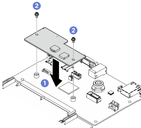
Figura 215. Instalação do Firmware e o módulo de segurança RoT
