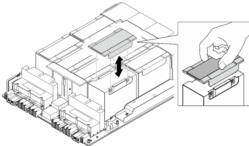
Figura 116. Instalação da tampa plástica
