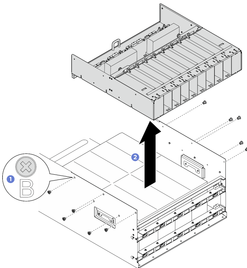
Figura 184. Remoção do Complexo de energia
