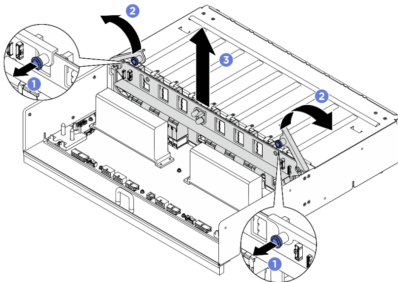
Figura 205. Remoção do Placa de interposição de PSU
