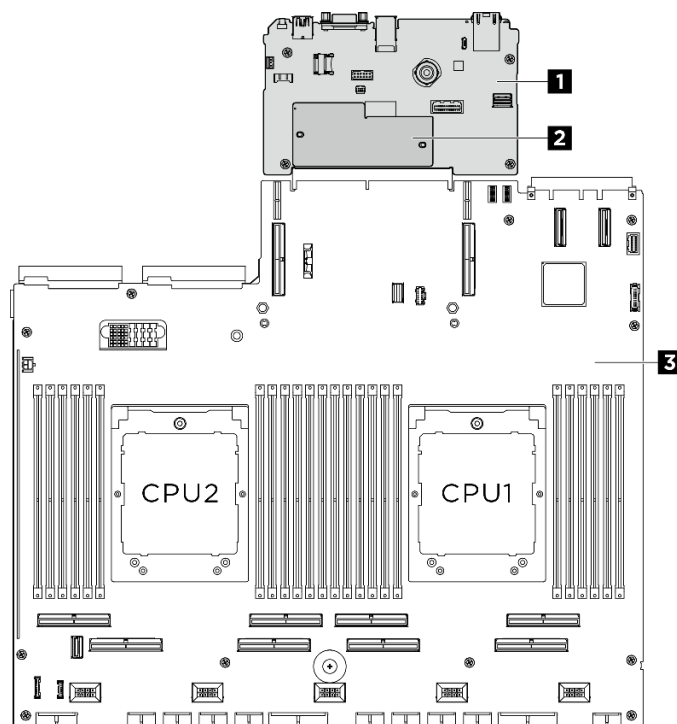
Figura 213. Layout do conjunto de placa-mãe
