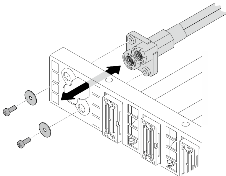
Figura 176. Remoção do cabo de alimentação
