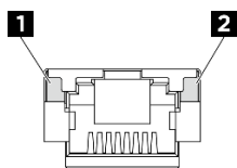
Figura 268. LEDs da Porta de gerenciamento de sistemas XCC (10/100/1.000 Mbps RJ-45)
