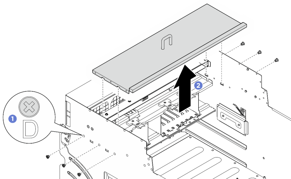
Figura 123. Remoção da tampa de E/S
