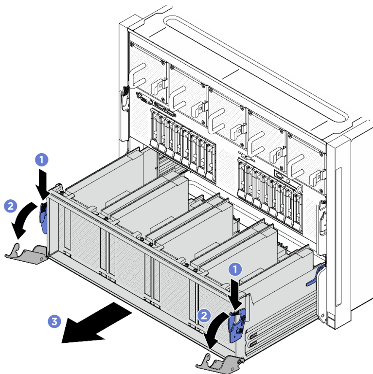
Figura 180. Remoção do Alternador do comutador PCIe para a posição de parada
