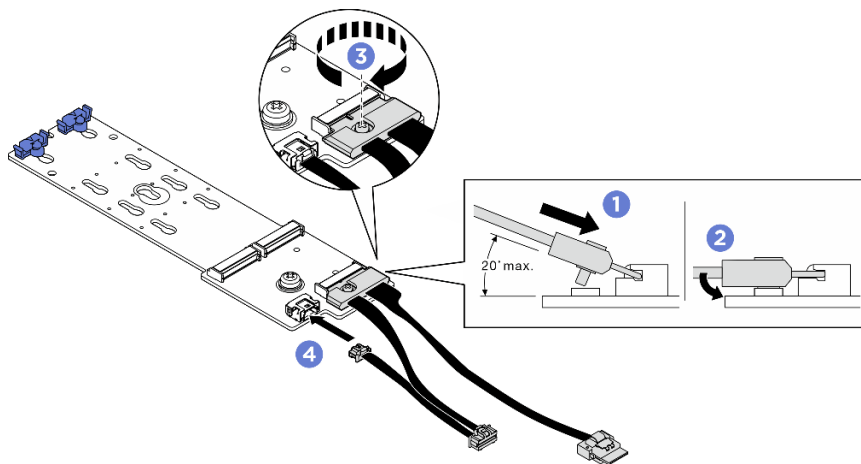
Figura 128. Conexão do cabo do backplane M.2
