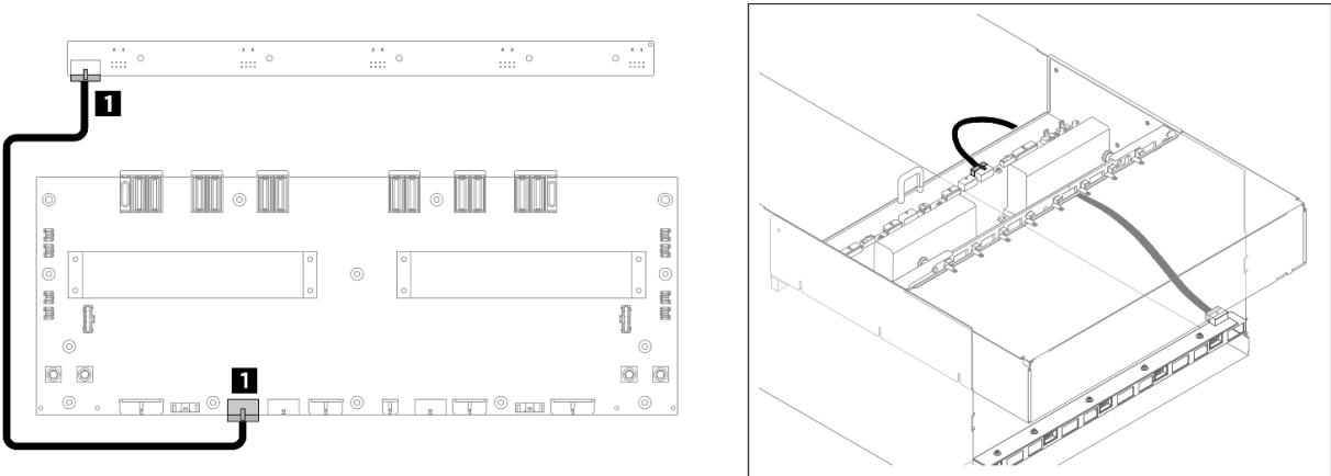
Figura 251. Roteamento de cabos da placa de controle do ventilador traseiro (inferior)
