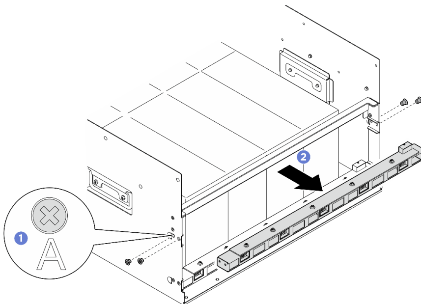
Figura 61. Remoção do conjunto de placa de controle do ventilador traseiro
