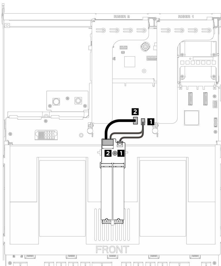
Figura 198. Conexão do cabo do backplane M.2
