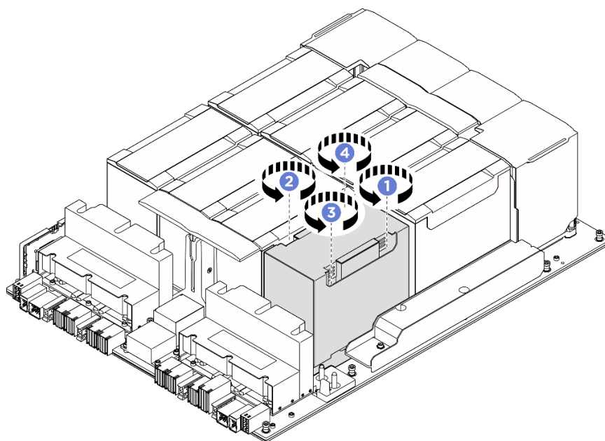
Figura 115. Sequência de aperto dos parafusos
