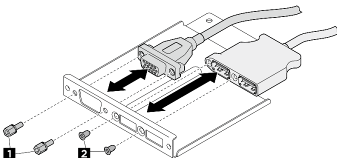
Figura 164. Remoção dos cabos do módulo de E/S frontal
