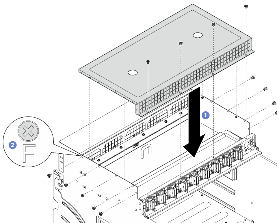
Figura 47. Instalação da tampa do cabo
