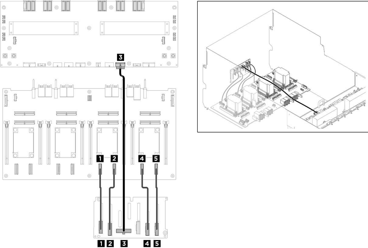
Figura 246. Roteamento de cabos do backplane 2
