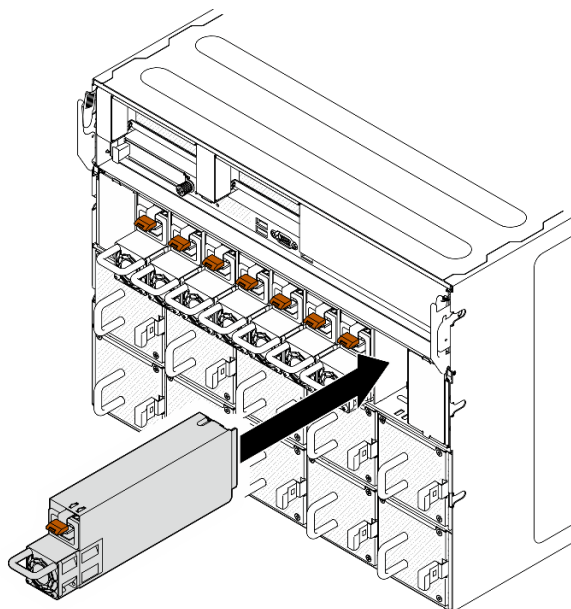
Figura 195. Instalação da unidade de fonte de alimentação
