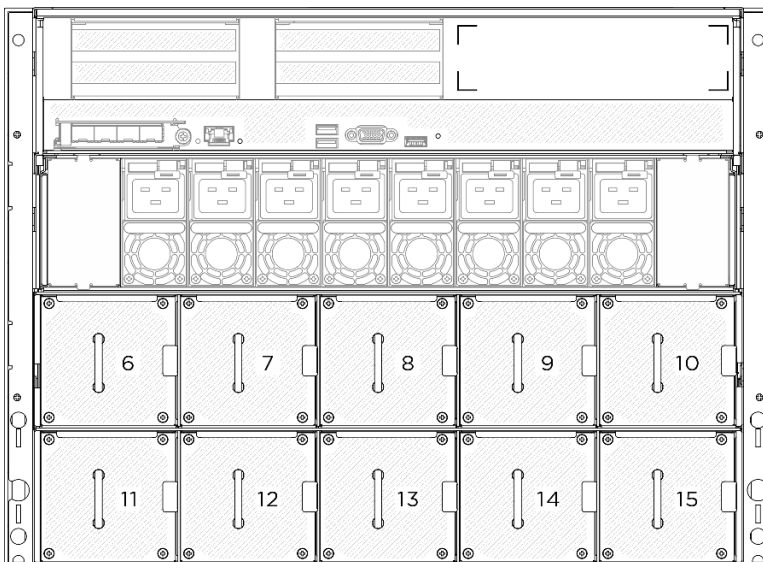
Figura 51. Numeração do ventilador traseiro
