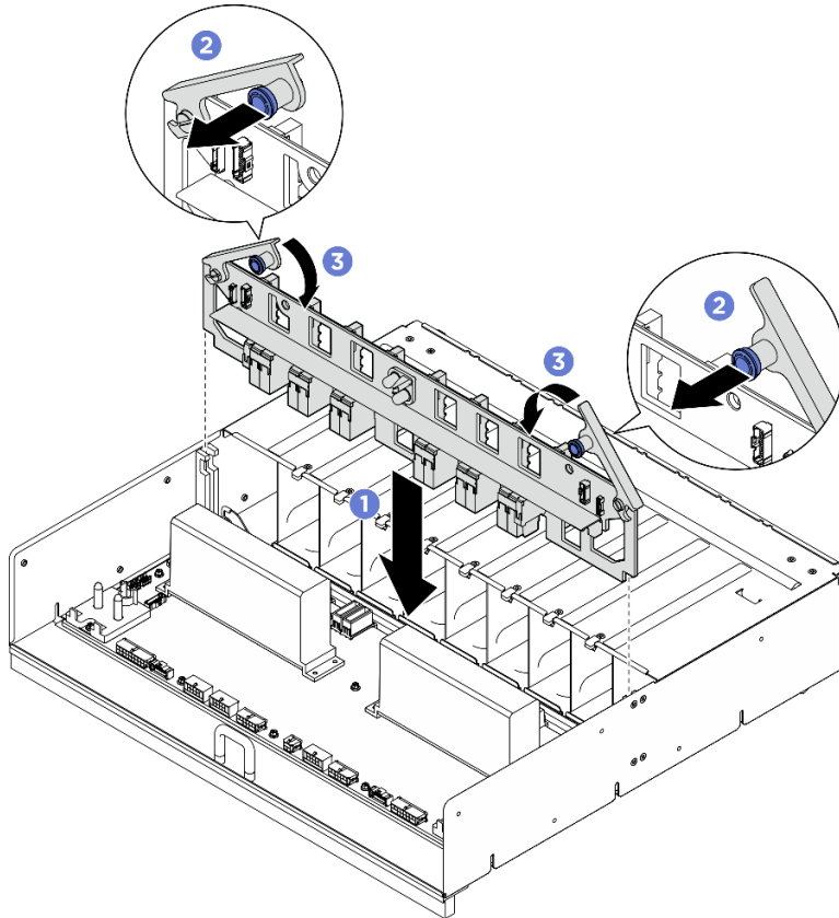
Figura 212. Instalação do Placa de interposição de PSU
