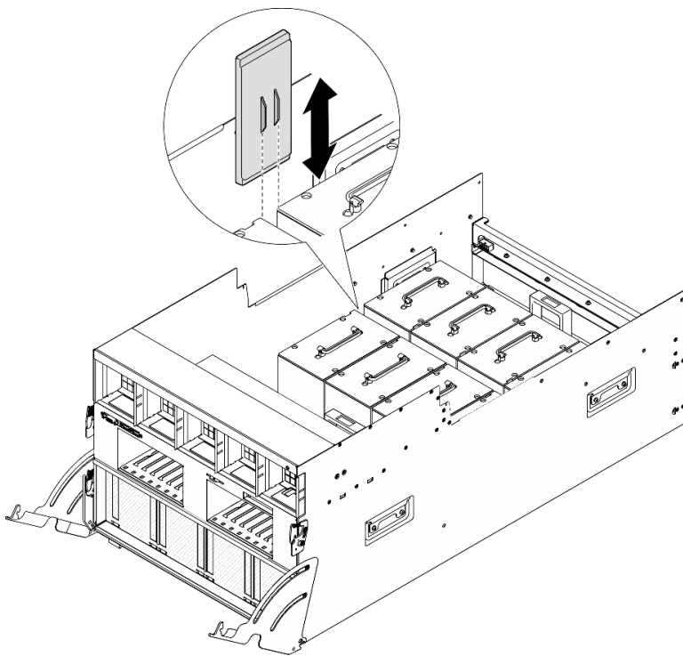
Figura 71. Remoção do duto de ar da GPU
