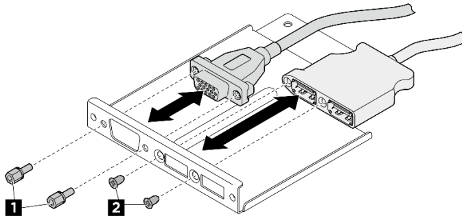
Figura 172. Instalação dos cabos do módulo de E/S frontal
