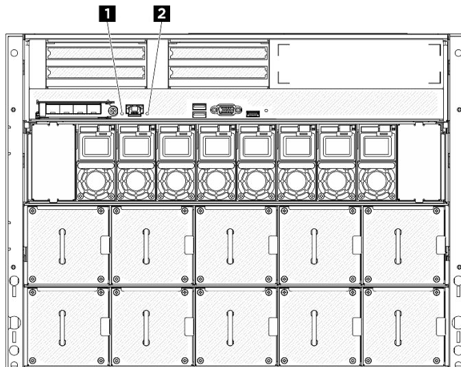
Figura 267. LEDs do sistema na vista traseira
