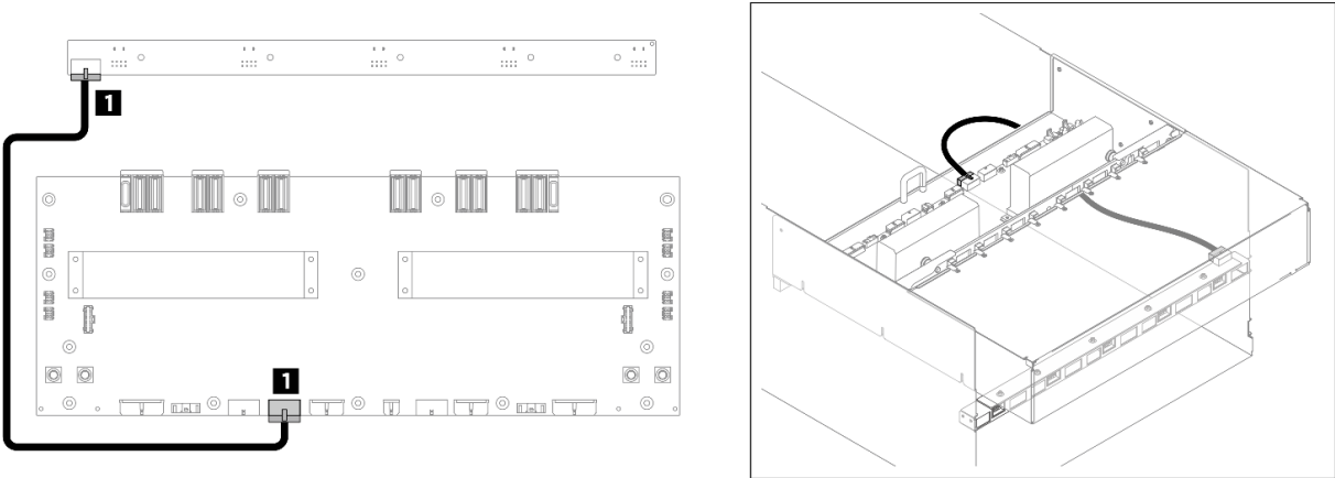
Figura 250. Roteamento de cabos da placa de controle do ventilador traseiro (superior)
