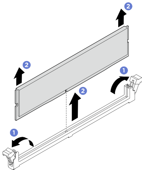
Figura 135. Remoção do módulo de memória
