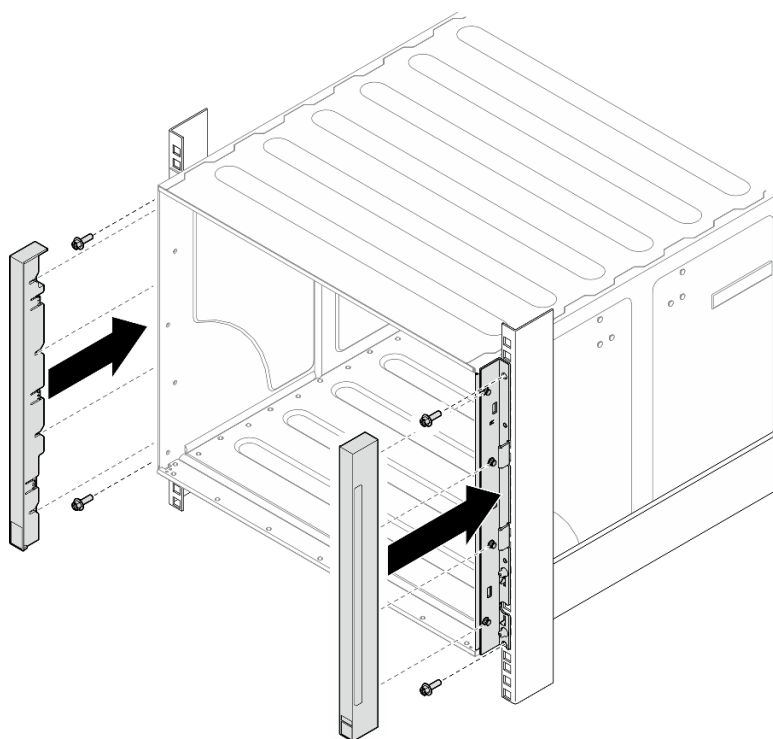
Figura 30. Instalação da tampa do EIA
