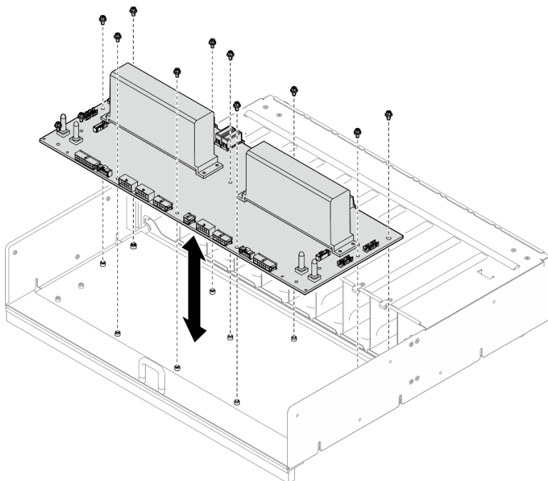
Figura 188. Instalação da placa de distribuição de energia
