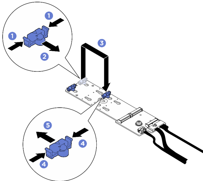
Figura 131. Ajuste do retentor do backplane M.2
