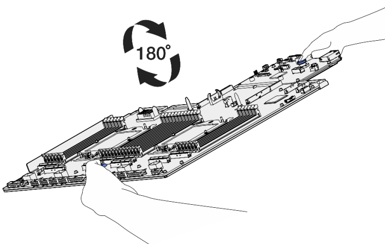
Figura 219. Girando o conjunto de placa-mãe para baixo
