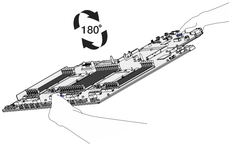
Figura 228. Girando o conjunto de placa-mãe para baixo
