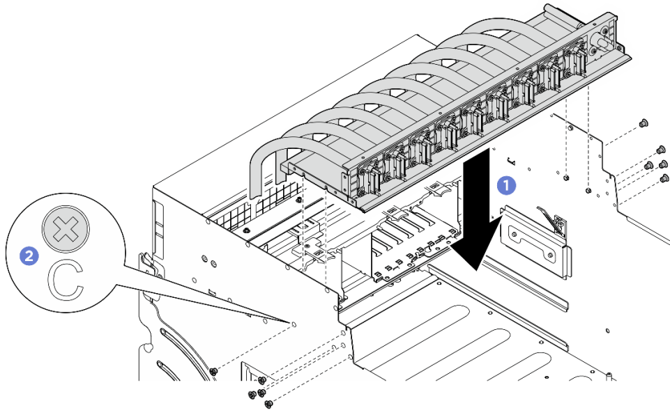
Figura 171. Instalação do Conjunto de cabos do comutador PCIe frontal
