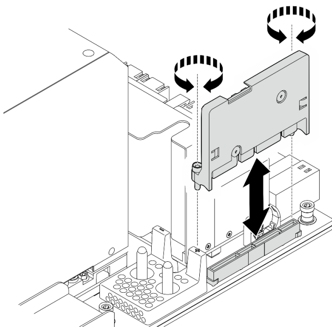
Figura 120. Instalação da placa HMC
