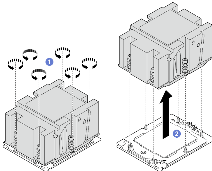
Figura 200. Remoção do dissipador de calor
