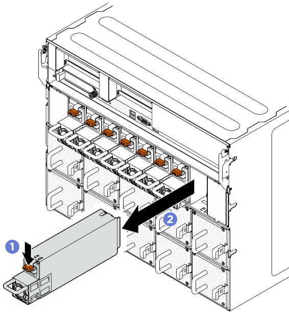
Figura 193. Remoção da unidade de fonte de alimentação
