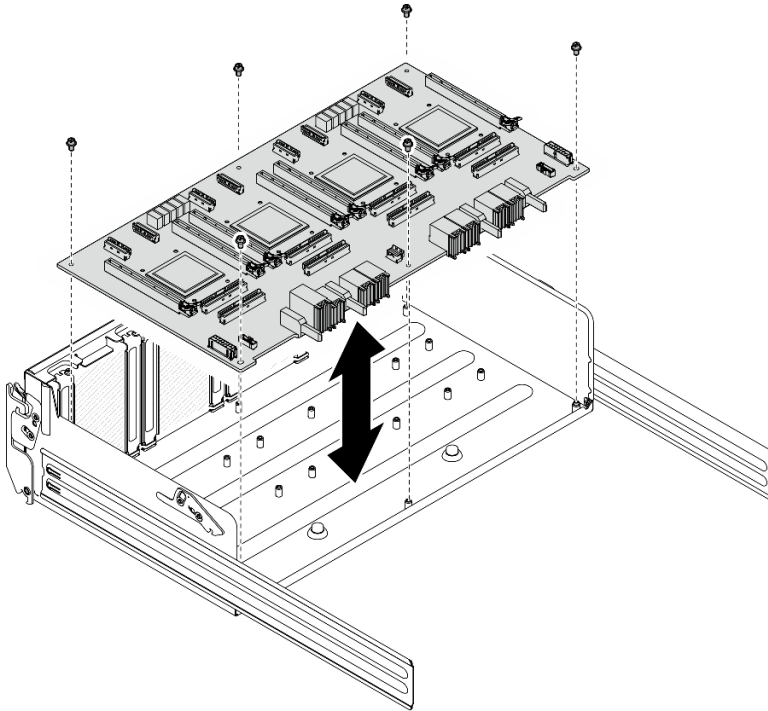
Figura 160. Instalação do Placa de comutador PCIe
