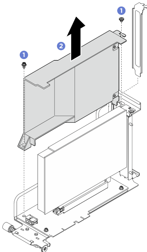
Figura 148. Remoção do defletor de ar da placa riser PCIe
