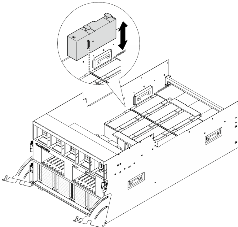
Figura 69. Remoção do duto de ar da GPU
