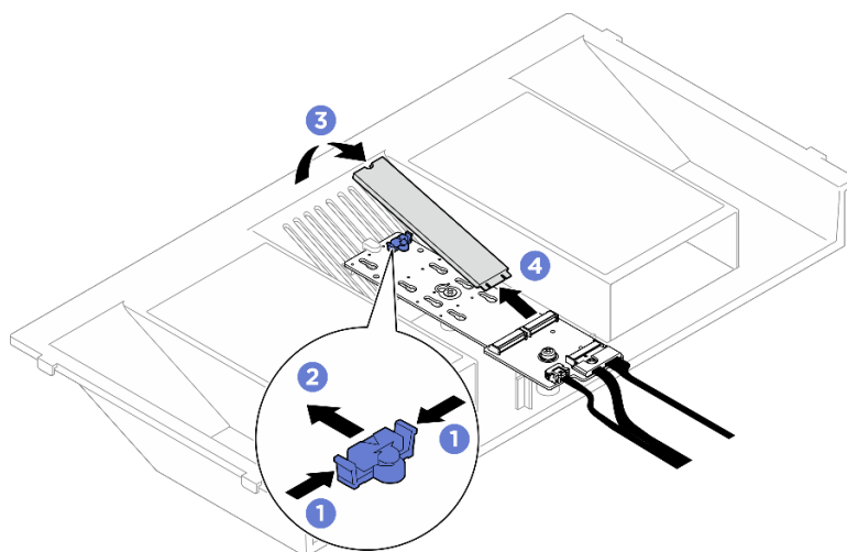
Figura 125. Remoção da unidade M.2
