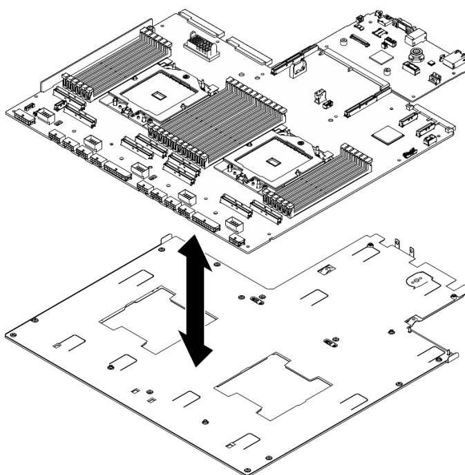
Figura 223. Desmontagem do conjunto da placa-mãe
