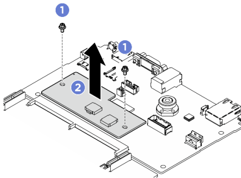
Figura 214. Remoção do Firmware e o módulo de segurança RoT
