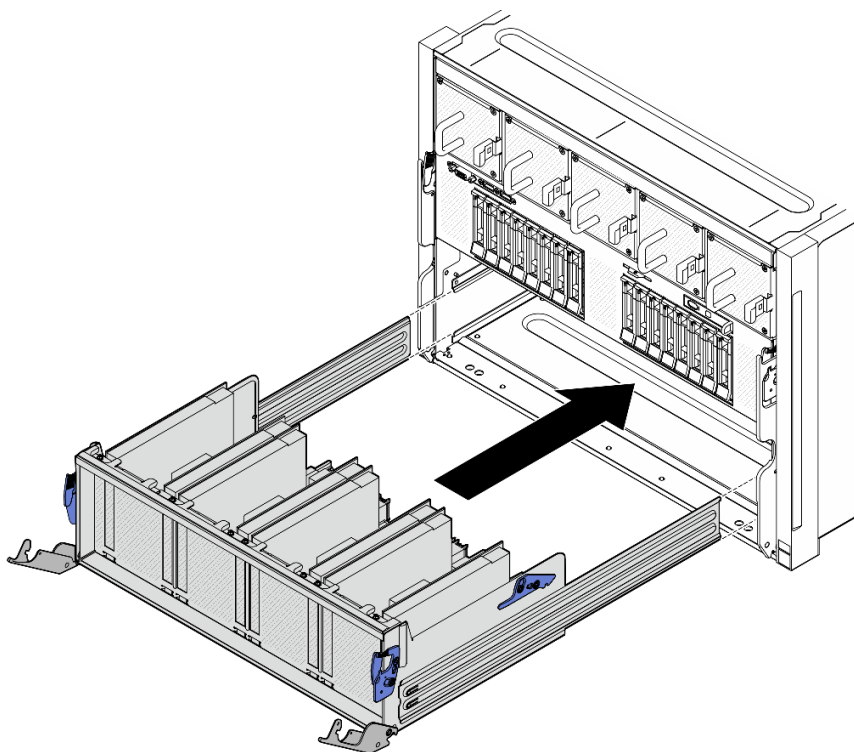
Figura 182. Instalação do Alternador do comutador PCIe na posição de parada
