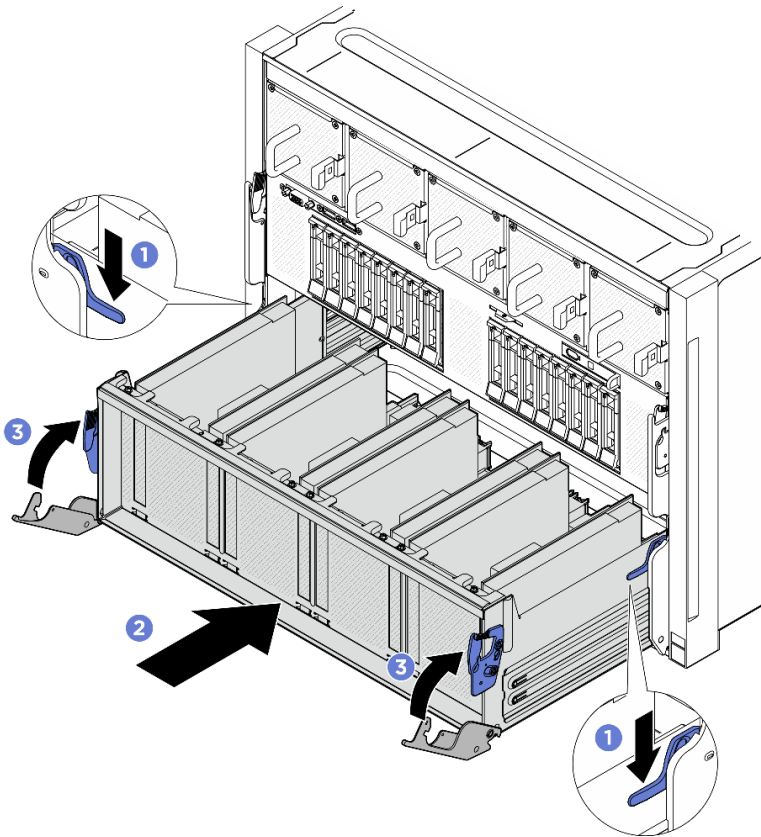
Figura 93. Instalação do Alternador do comutador PCIe no Alternador de GPU 8U
