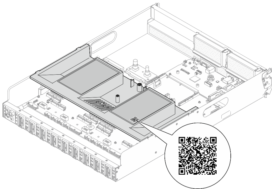
Figura 16. Etiqueta de serviço e código QR
