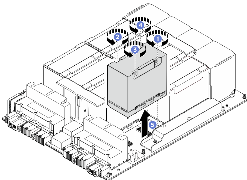
Figura 113. Remoção do Módulo de GPU e dissipador de calor
