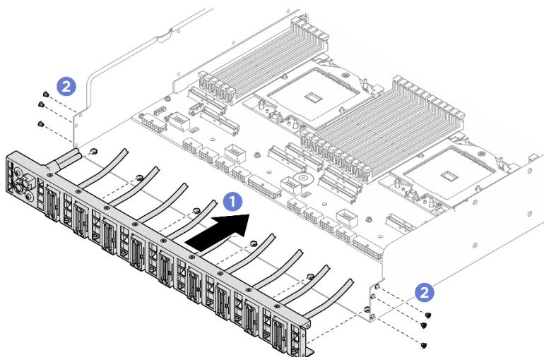
Figura 179. Instalação do Conjunto de cabos do comutador PCIe traseiro
