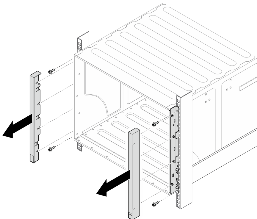
Figura 20. Remoção da tampa do EIA
