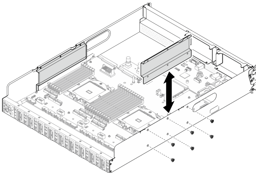
Figura 216. Remoção do guia de cabos
