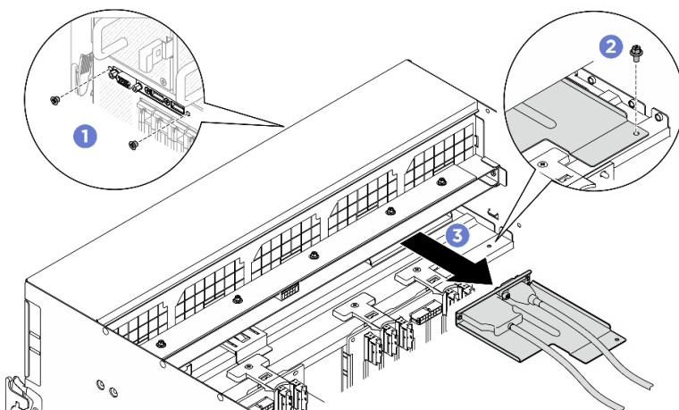
Figura 163. Remoção do módulo de E/S frontal
