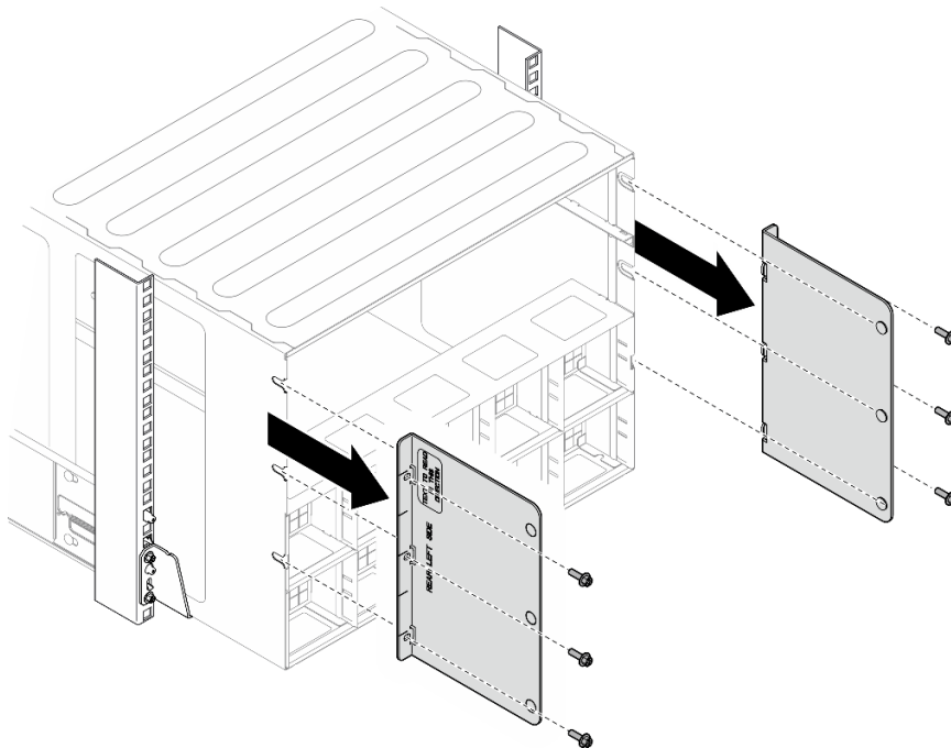
Figura 18. Remoção do suporte de apoio superior
