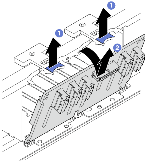
Figura 38. Remoção do painel traseiro da unidade de 2,5 polegadas
