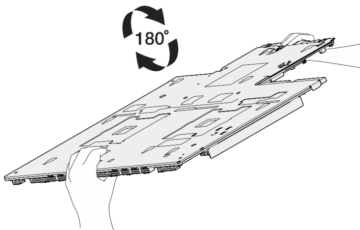
Figura 274. Girando o conjunto de placa-mãe lado direito para cima
