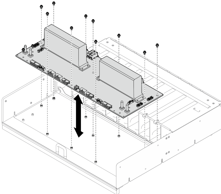
Figura 187. Remoção da placa de distribuição de energia
