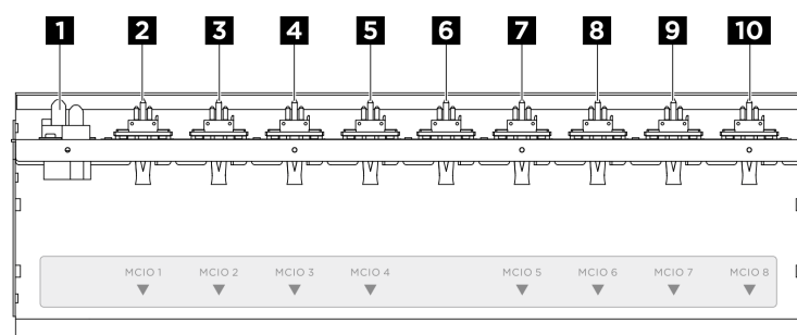
Figura 239. Cabos do conjunto de cabos do comutador PCIe frontal
