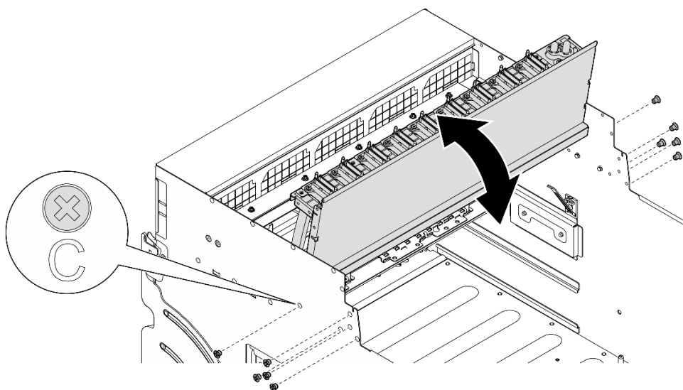
Figura 109. Virando o conjunto de cabos do comutador PCIe frontal
