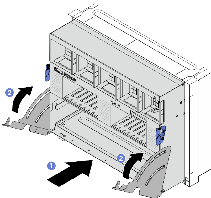
Figura 45. Instalação do Alternador de GPU 8U
