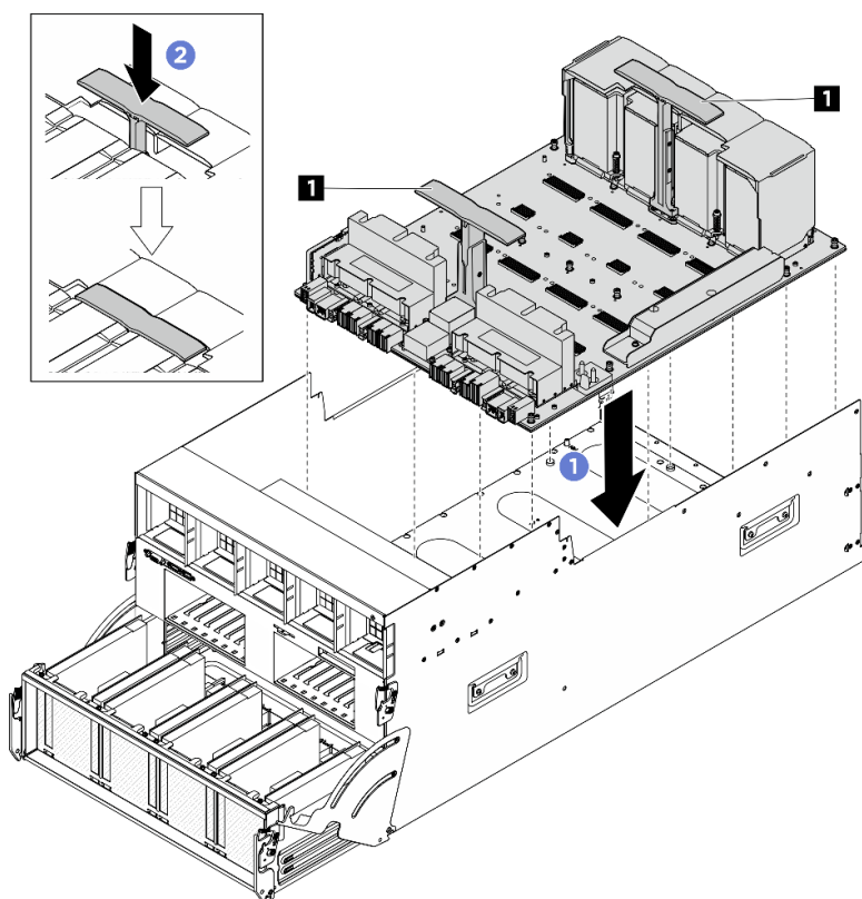
Figura 79. Instalação do Placa-base da GPU
