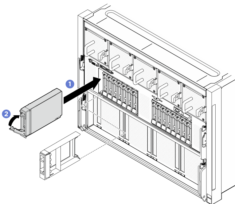
Figura 36. Instalação de uma unidade hot-swap de 2,5 polegadas
