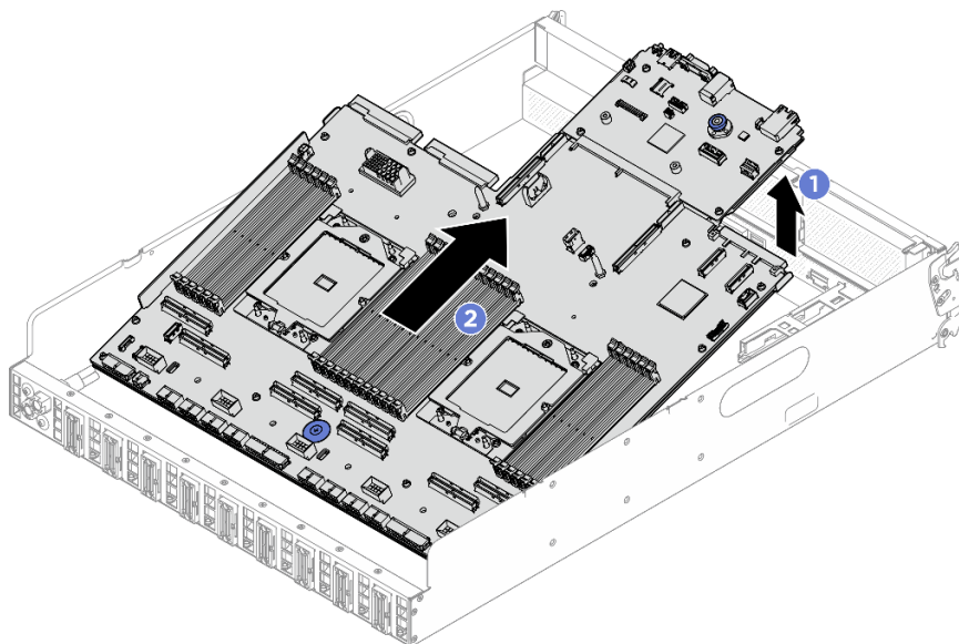
Figura 271. Remoção do conjunto de placa-mãe
