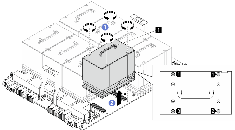
Figura 117. Remoção do Módulo de GPU e dissipador de calor
