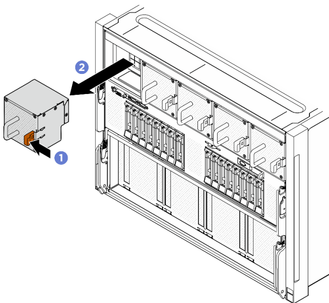
Figura 52. Remoção do ventilador hot swap
