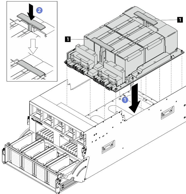
Figura 90. Instalação do Complexo da GPU
