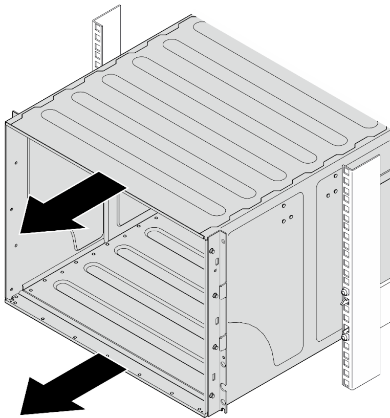
Figura 21. Deslizando o chassi
