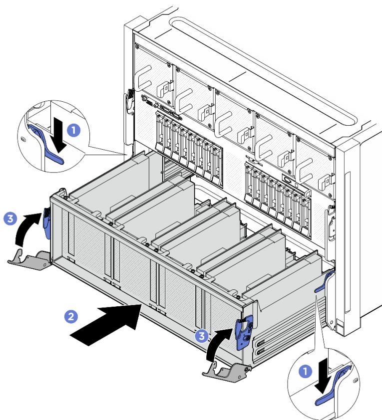
Figura 183. Instalação do Alternador do comutador PCIe no Alternador de GPU 8U
