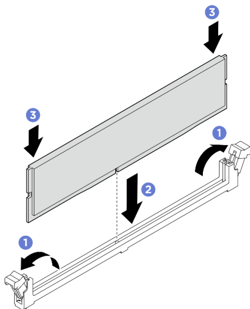
Figura 137. Instalação do módulo de memória
