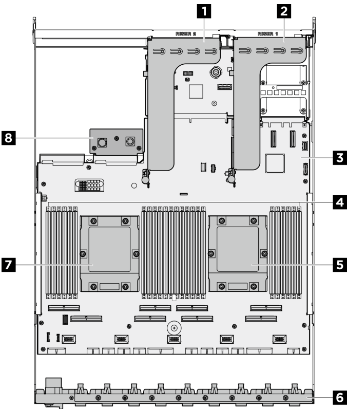
Figura 7. Vista superior do Alternador de cálculo 2U
