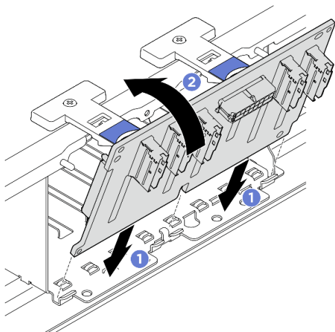
Figura 40. Instalação do painel traseiro da unidade de 2,5 polegadas
