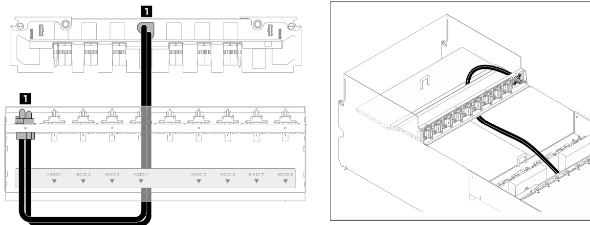
Figura 261. Roteamento de cabos da Placa de interface de alimentação
