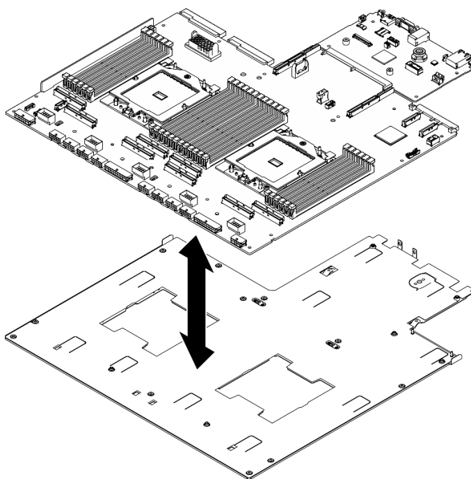
Figura 276. Desmontagem do conjunto da placa-mãe
