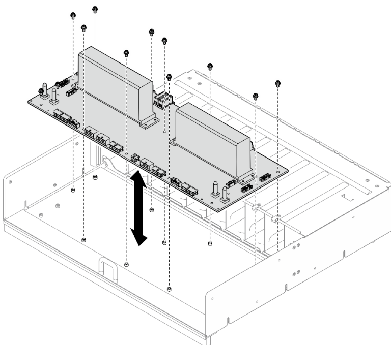
Figura 207. Remoção da placa de distribuição de energia
