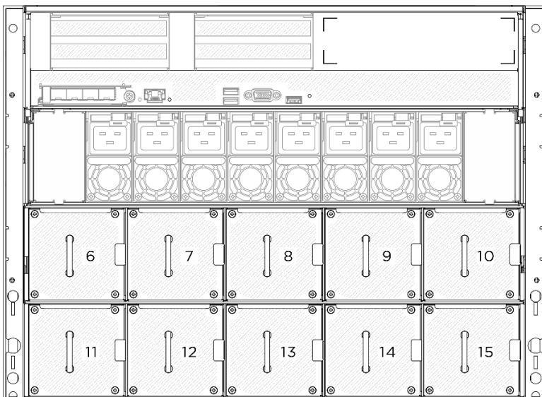
Figura 54. Numeração do ventilador traseiro
