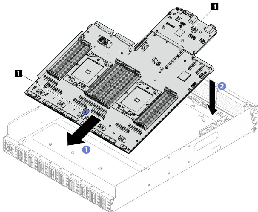
Figura 231. Instalação do conjunto de placa-mãe
