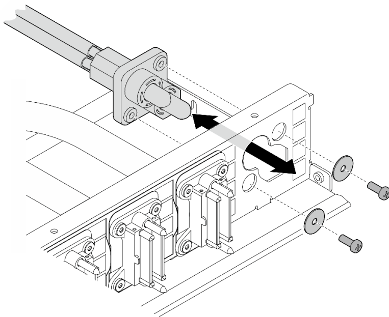
Figura 170. Instalação do cabo de alimentação
