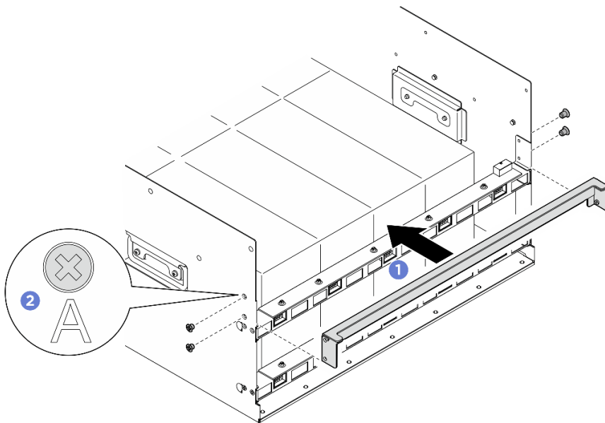
Figura 103. Instalação do suporte de apoio traseiro
