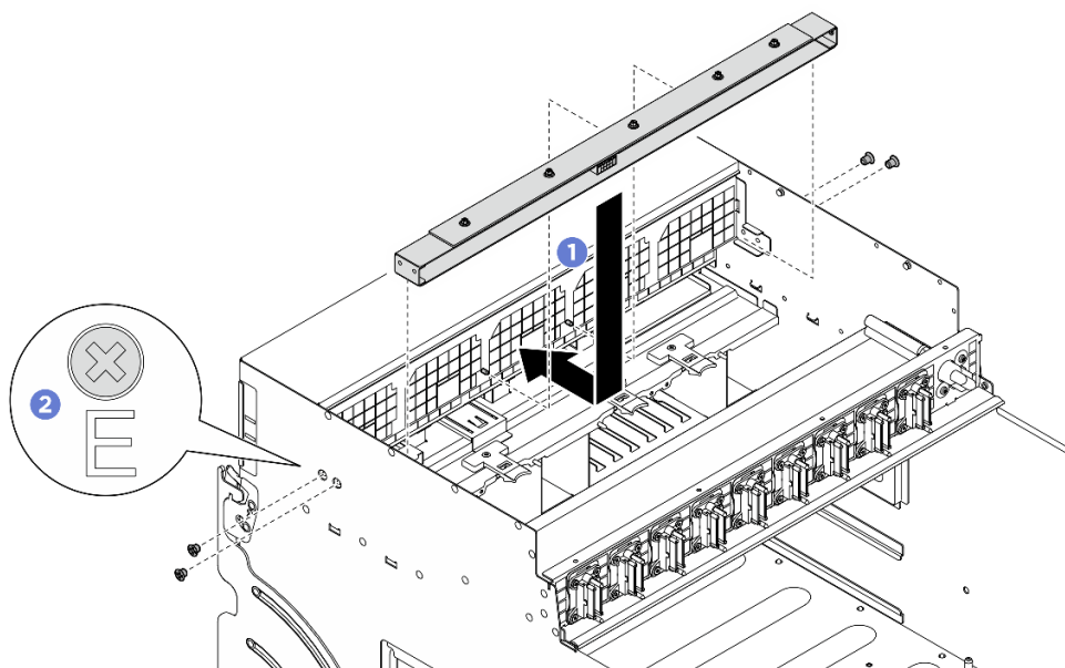
Figura 59. Instalação do conjunto de placa de controle do ventilador frontal
