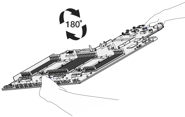
Figura 272. Girando o conjunto de placa-mãe para baixo
