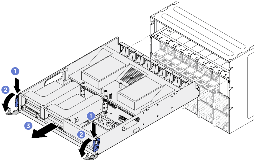
Figura 42. Remoção do Alternador de cálculo 2U
