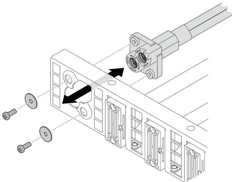
Figura 178. Instalação do cabo de alimentação
