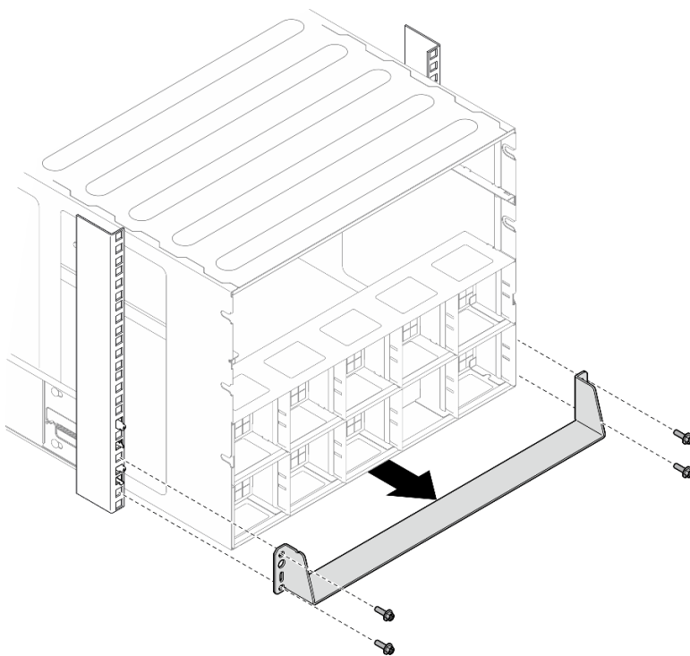
Figura 19. Remoção do suporte de apoio inferior
