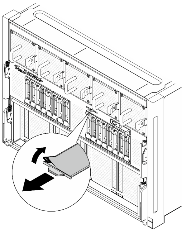
Figura 15. Etiqueta de acesso à rede do Lenovo XClarity Controller na guia de informações removível
