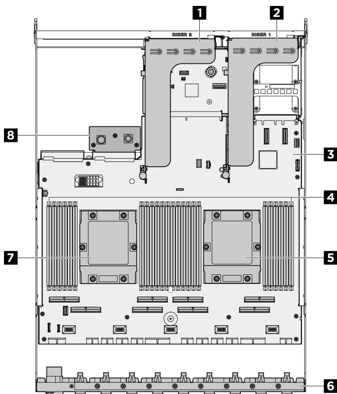
圖例 7. 2U 運算滑動箱俯視圖
