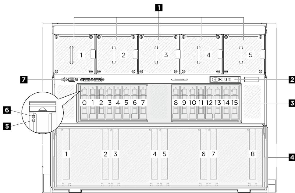
圖例 2. 正面圖
