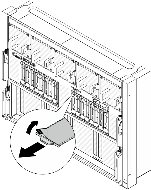
圖例 19. 拉出式資訊標籤上的 Lenovo XClarity Controller 網路存取標籤
