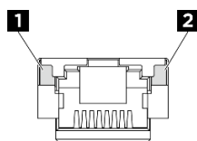
圖例 16. XCC 系統管理埠 (10/100/1000 Mbps RJ-45) LED
