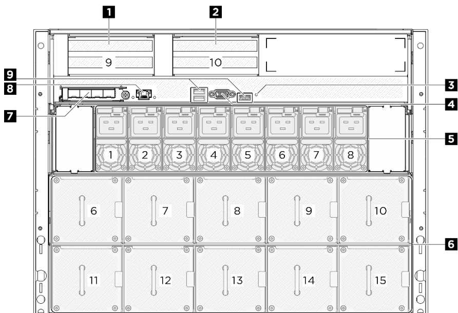
圖例 4. 背面圖
