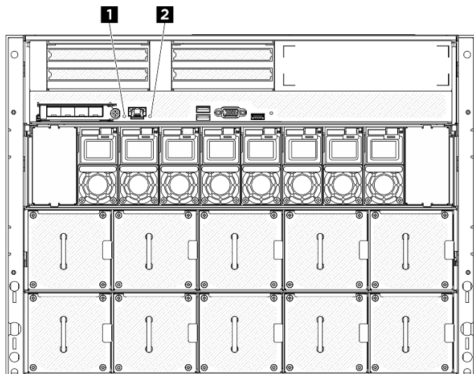
圖例 15. 背面圖上的系統 LED
