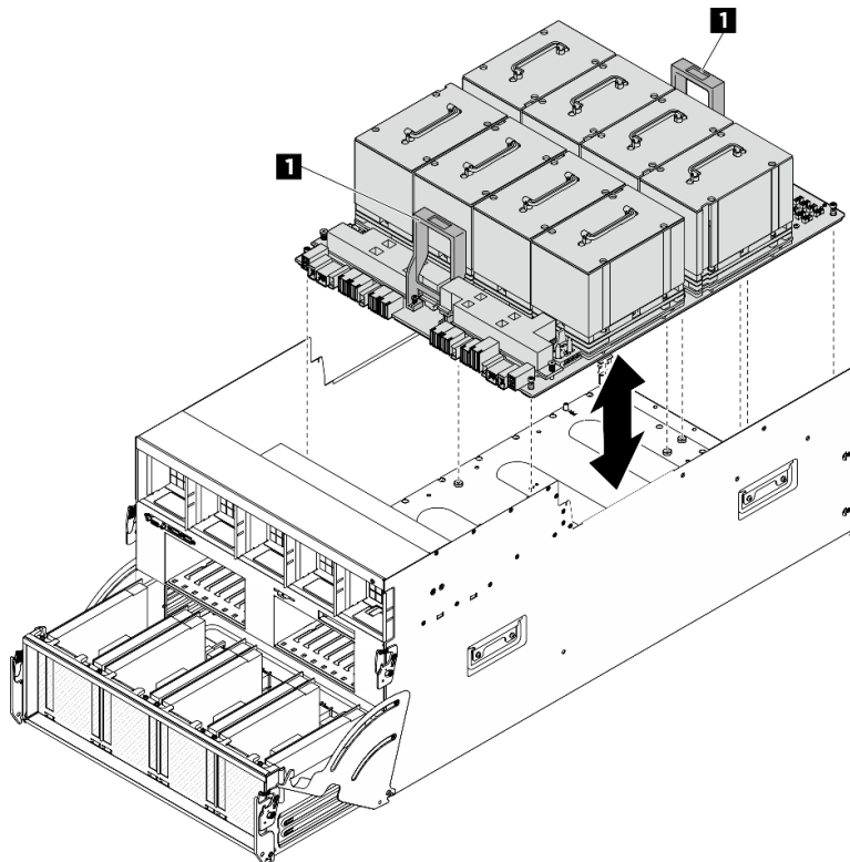
圖例 100. 安裝 GPU 複合體
