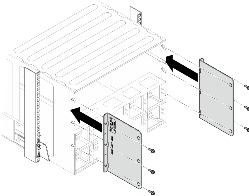
圖例 32. 安裝上支撐托架
