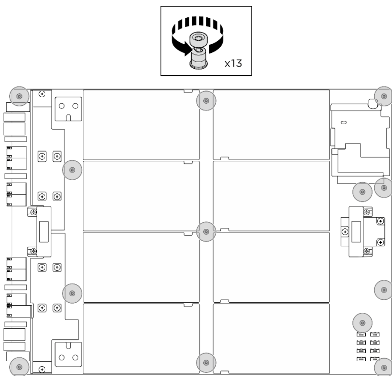
圖例 98. 卸下螺絲
