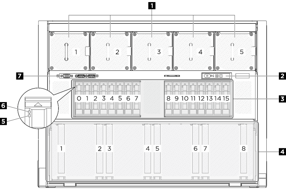
圖例 2. 正面圖
