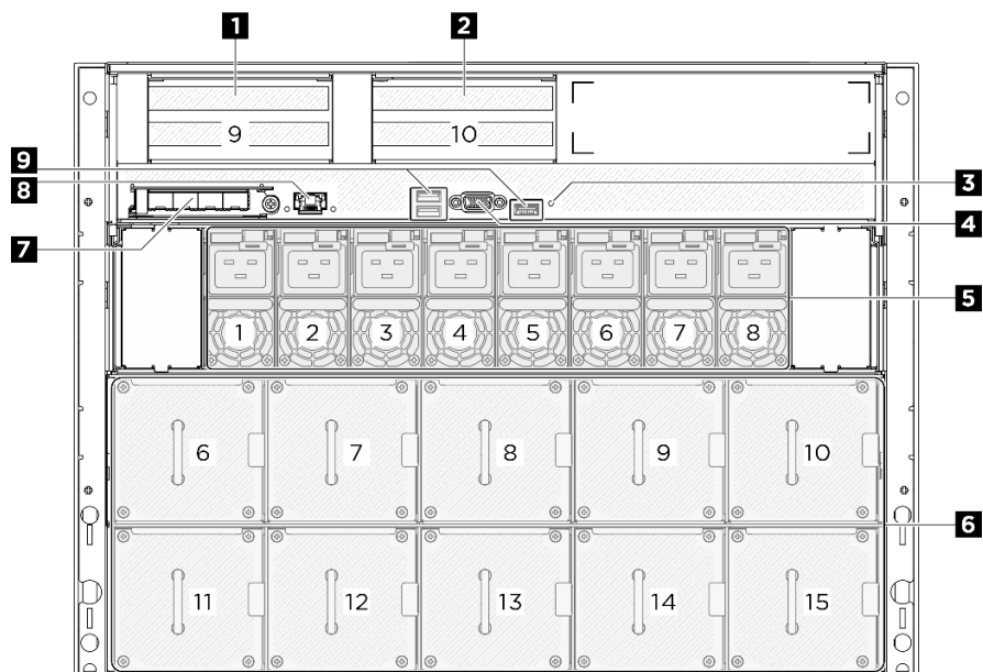
圖例 4. 背面圖
