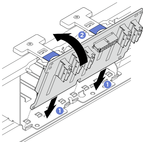
圖例 40. 2.5 吋硬碟背板安裝
