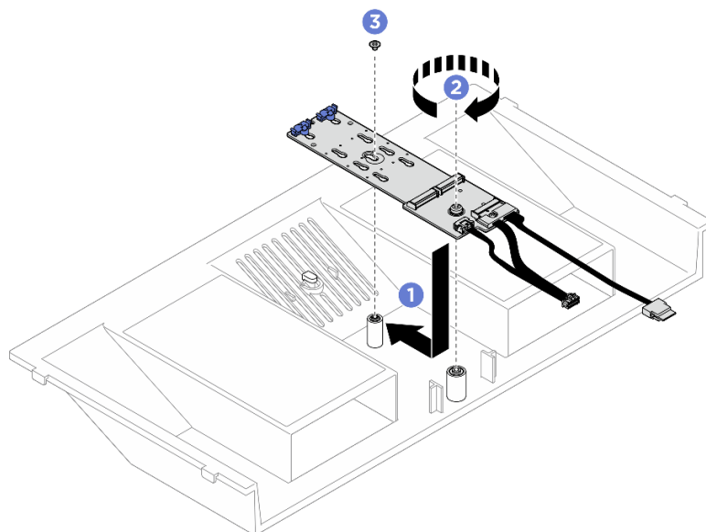
圖例 129. M.2 背板安裝
