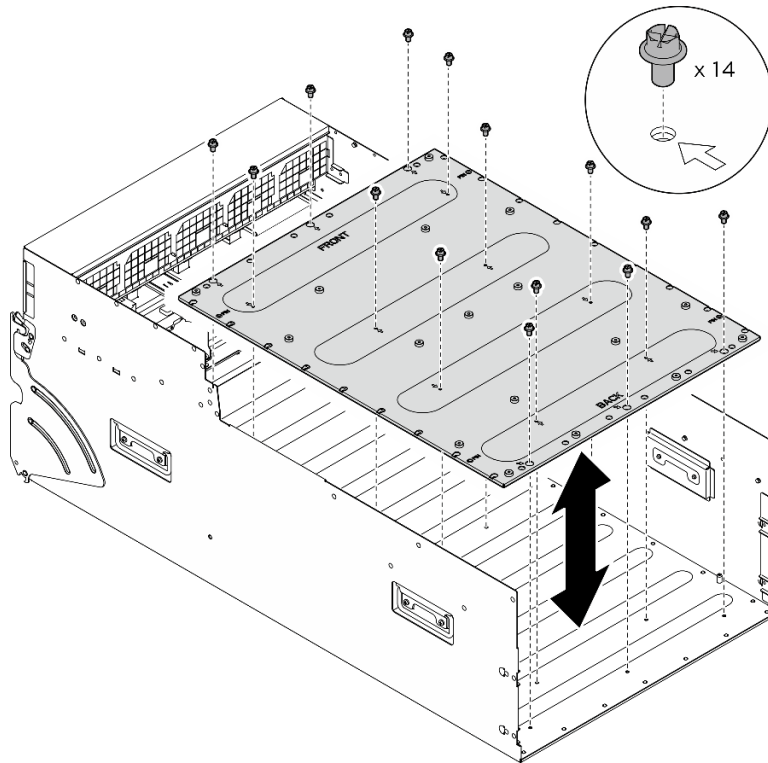
圖例 107. 卸下 GPU 複合體配接器板
