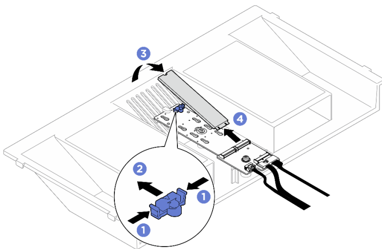
圖例 125. 卸下 M.2 硬碟
