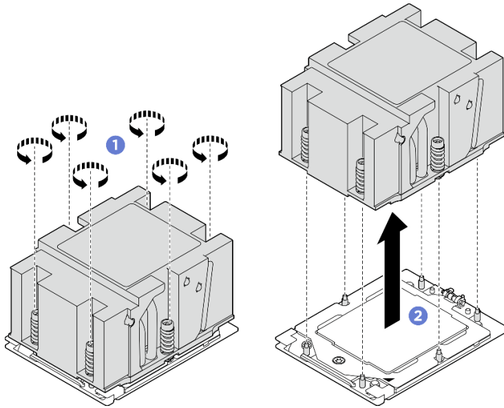
圖例 200. 卸下散熱槽
