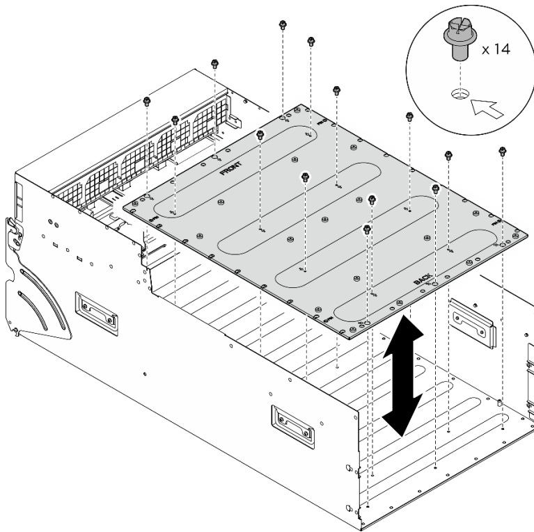
圖例 108. 安裝 GPU 複合體配接器板
