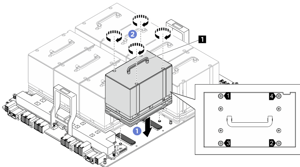
圖例 118. 安裝 GPU 和散熱槽模組
