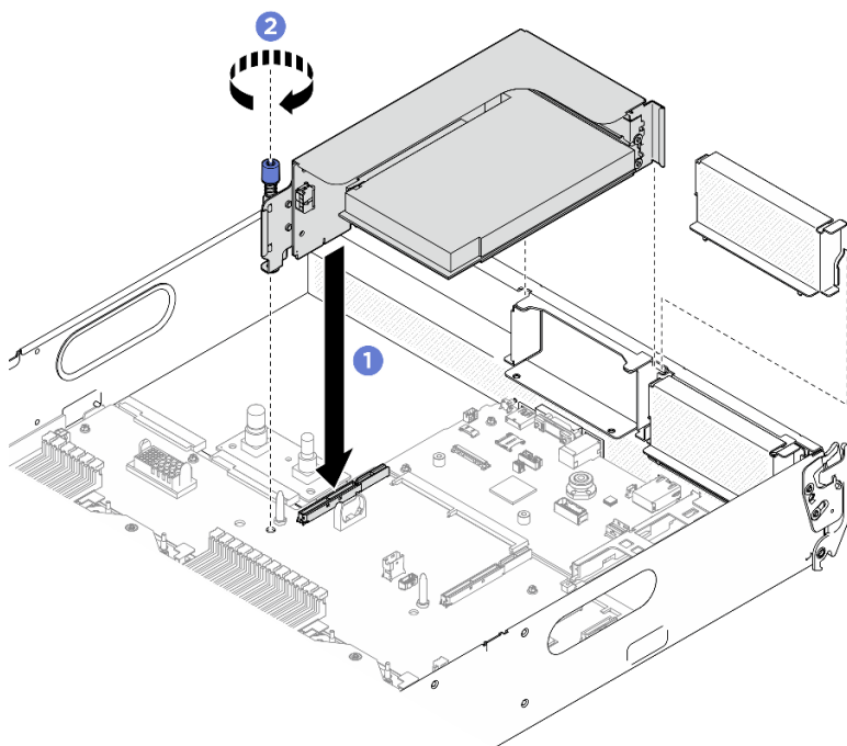
圖例 157. 安裝 PCIe 擴充卡組件
