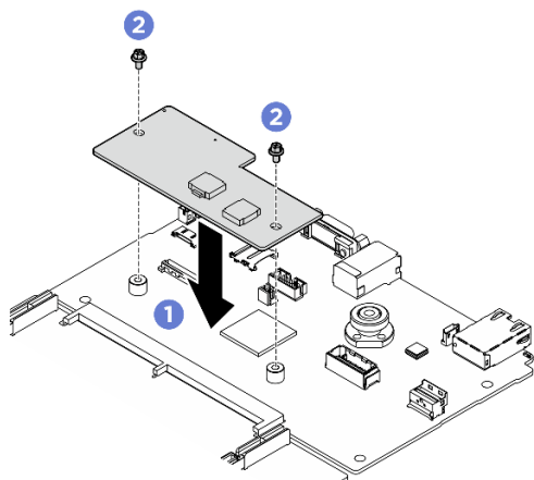
圖例 215. 安裝韌體和 RoT 安全模組
