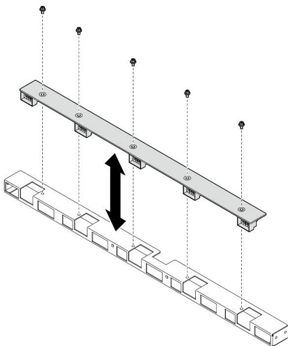
圖例 63. 安裝後方風扇控制板
