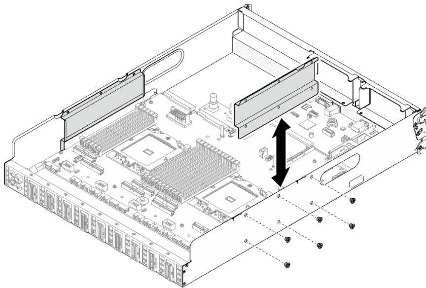
圖例 216. 卸下纜線導件
