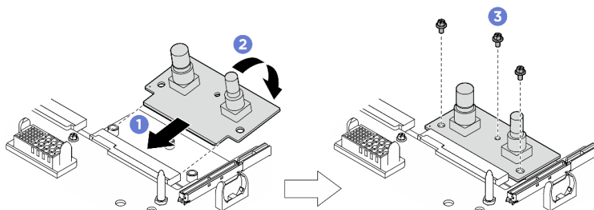
圖例 191. 電源介面板安裝
