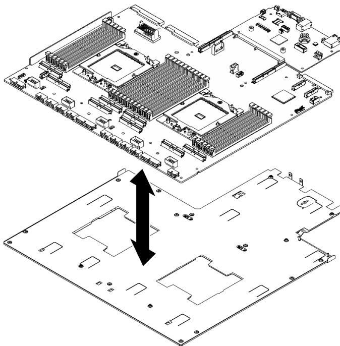
圖例 226. 安裝主機板組件
