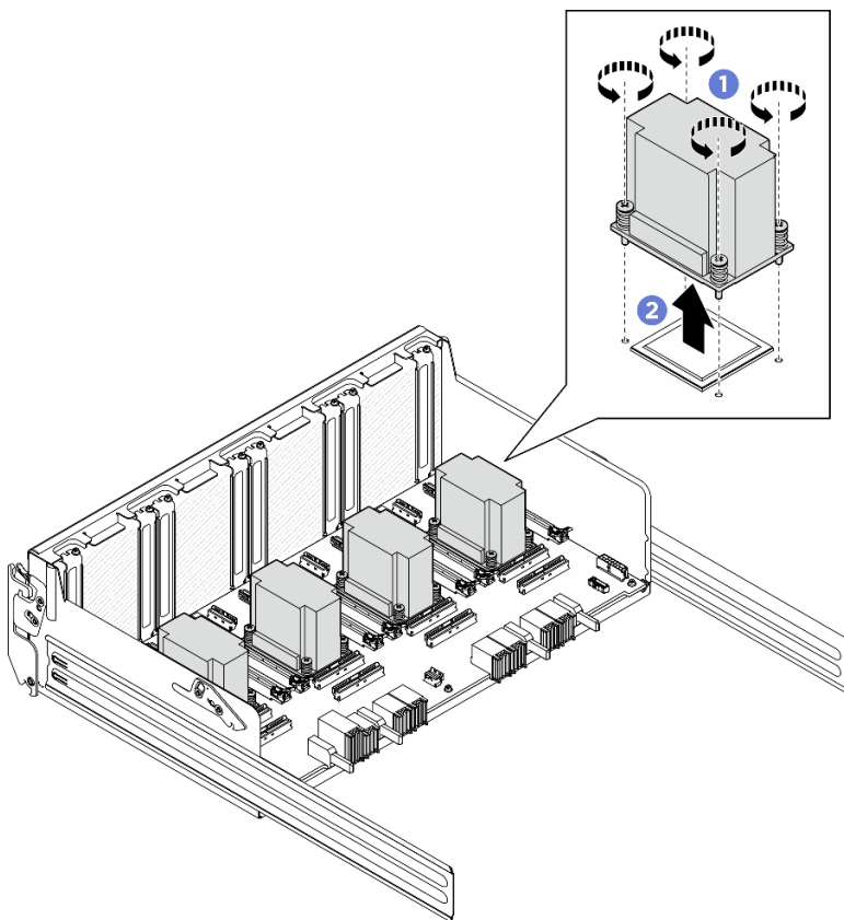
圖例 158. 卸下 PCIe 交換器板散熱槽
