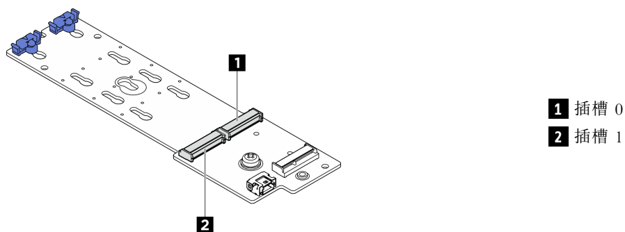
圖例 132. M.2 硬碟插槽
