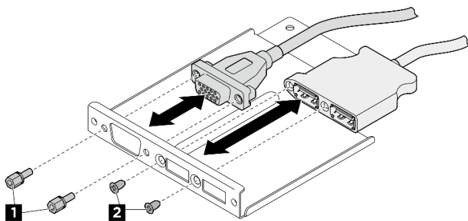
圖例 164. 卸下正面 I/O 模組纜線
