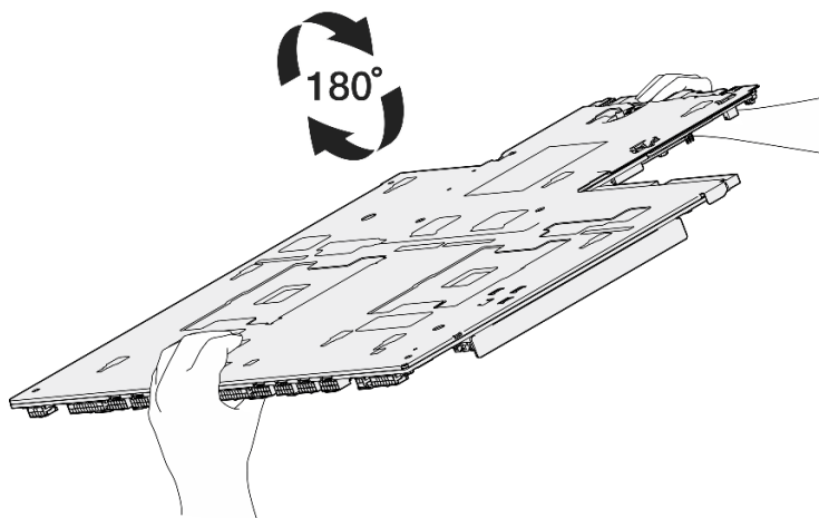
圖例 221. 將主機板組件轉至正面朝上
