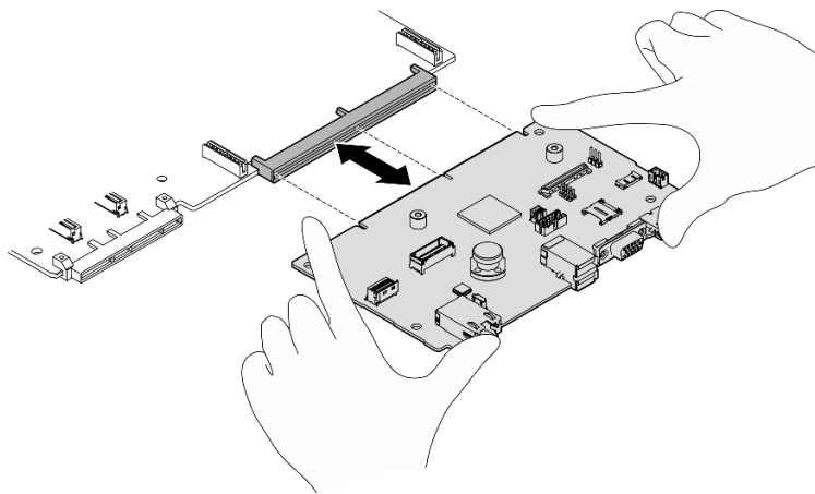
圖例 225. 安裝系統 I/O 板
