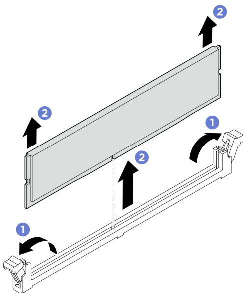
圖例 135. 卸下記憶體模組
