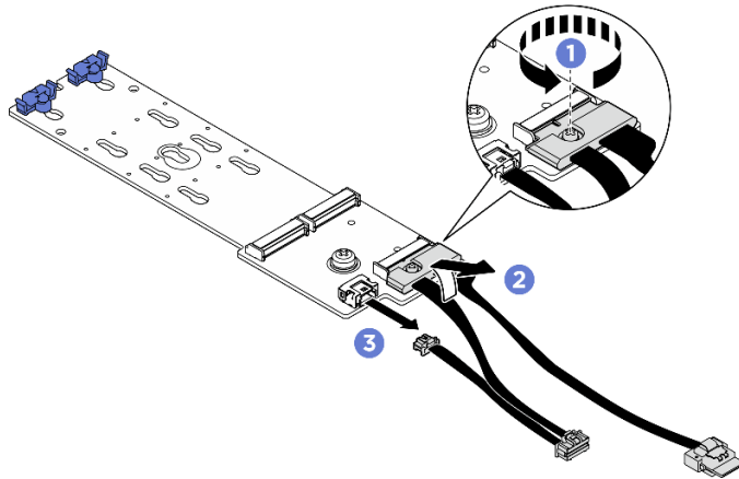
圖例 127. 拔除 M.2 背板纜線
