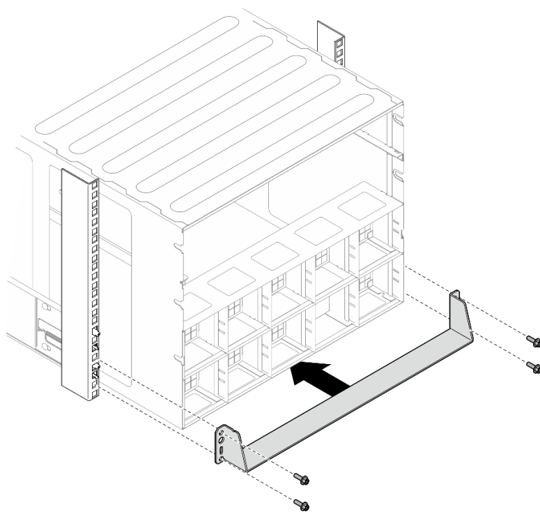
圖例 31. 安裝下支撐托架
