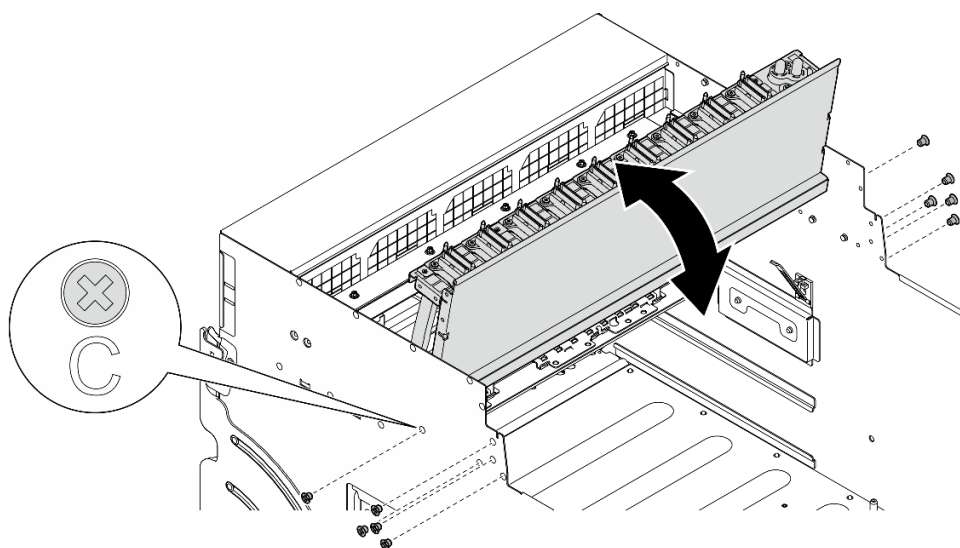
圖例 102. 翻轉前方 PCIe 交換器纜線載具
