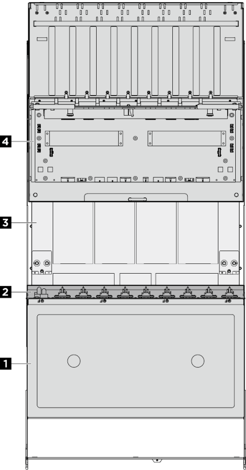
圖例 8. 8U GPU 滑動箱俯視圖
