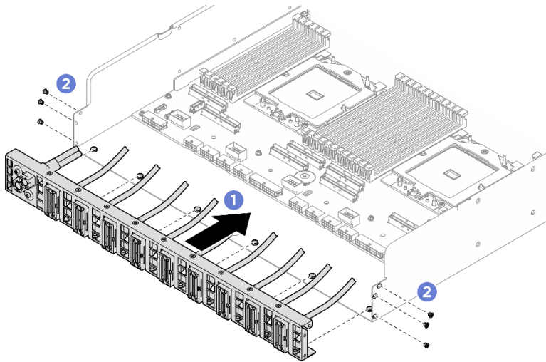
圖例 179. 安裝後方 PCIe 交換器纜線載具
