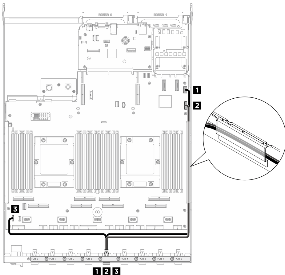
圖例 253. 正面 I/O 模組和整合式診斷面板纜線佈線
