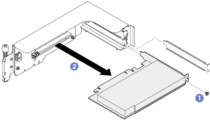
圖例 146. 卸下背面 PCIe 配接卡
