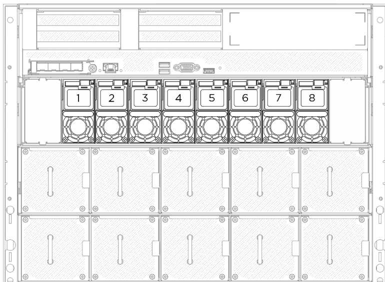
圖例 192. 電源供應器機槽編號
