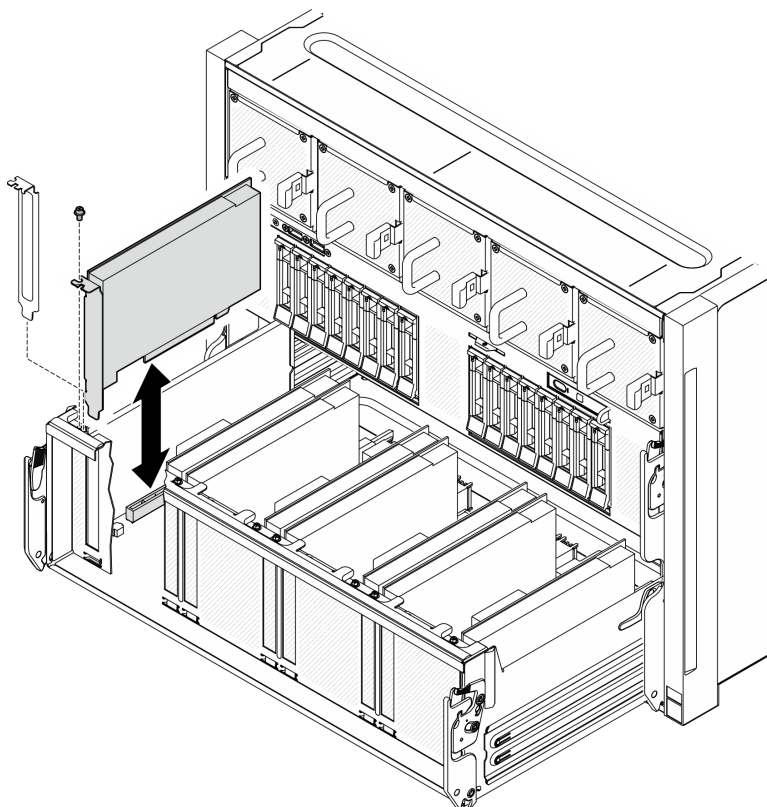
圖例 143. 卸下正面 PCIe 配接卡
