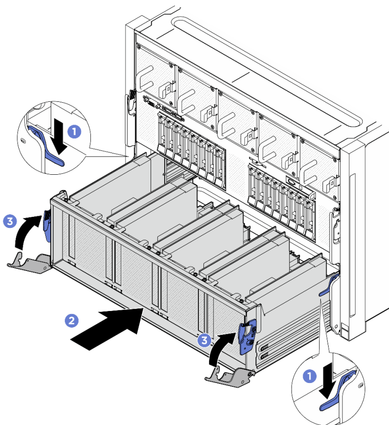
圖例 183. 將 PCIe 交換器滑動箱安裝到 8U GPU 滑動箱中
