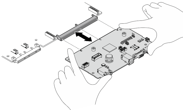
圖例 224. 卸下系統 I/O 板
