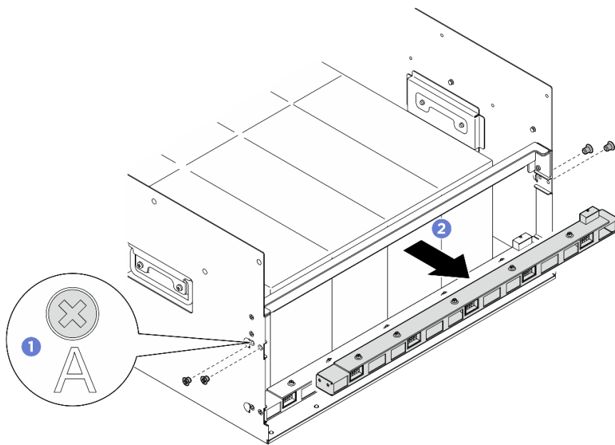
圖例 61. 卸下後方風扇控制板組件
