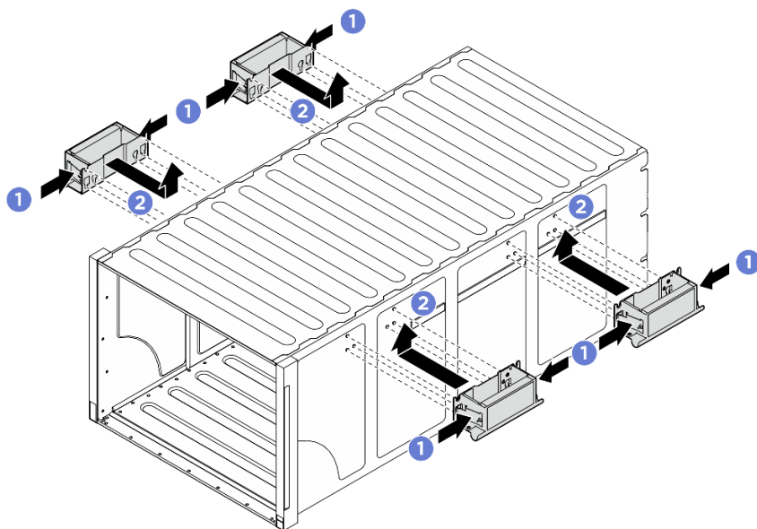
圖例 26. 安裝四個把手
