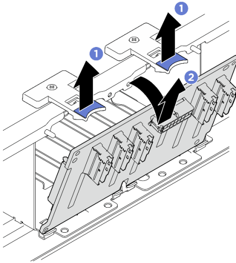
圖例 38. 卸下 2.5 吋硬碟背板
