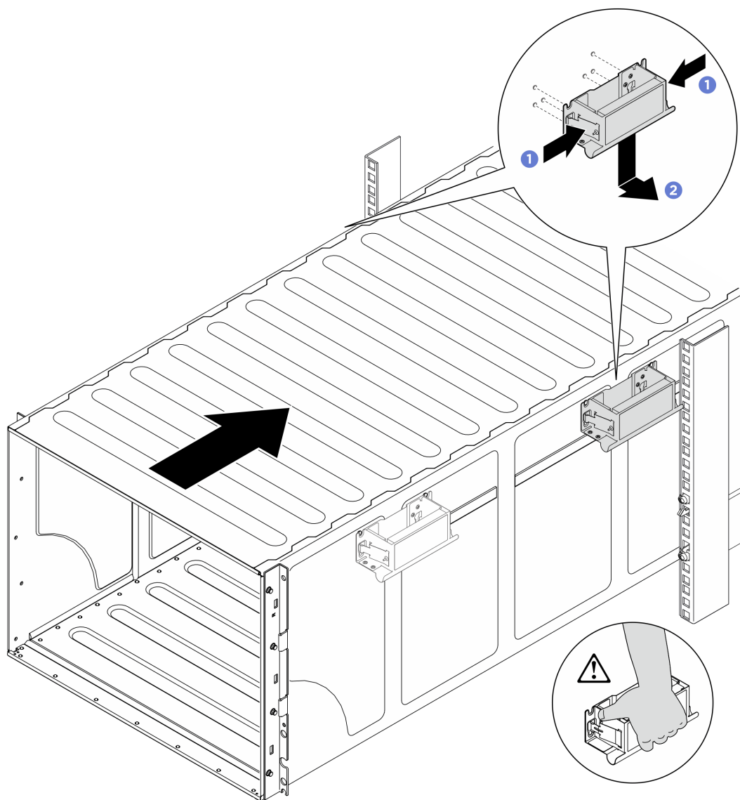
圖例 27. 卸下後把手
