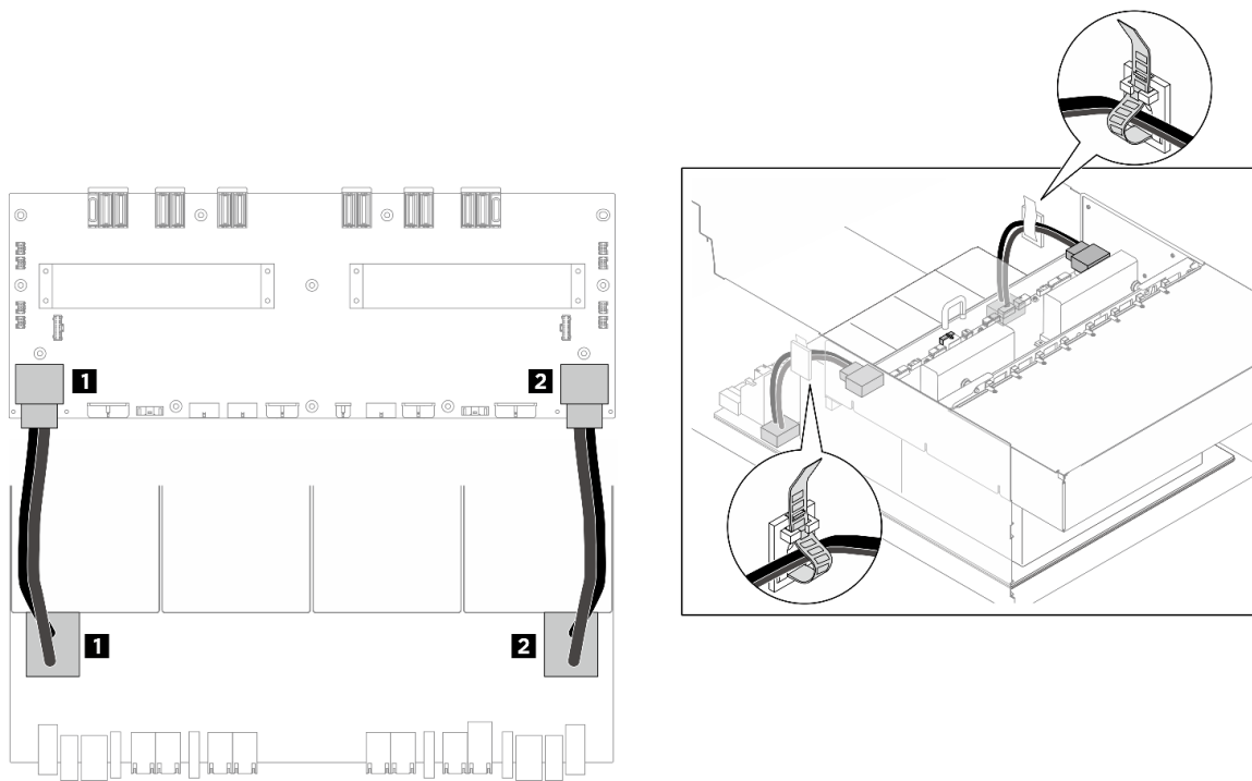
圖例 252. GPU 基板纜線佈線
