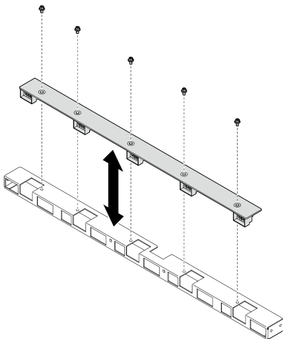
圖例 58. 安裝前方風扇控制板
