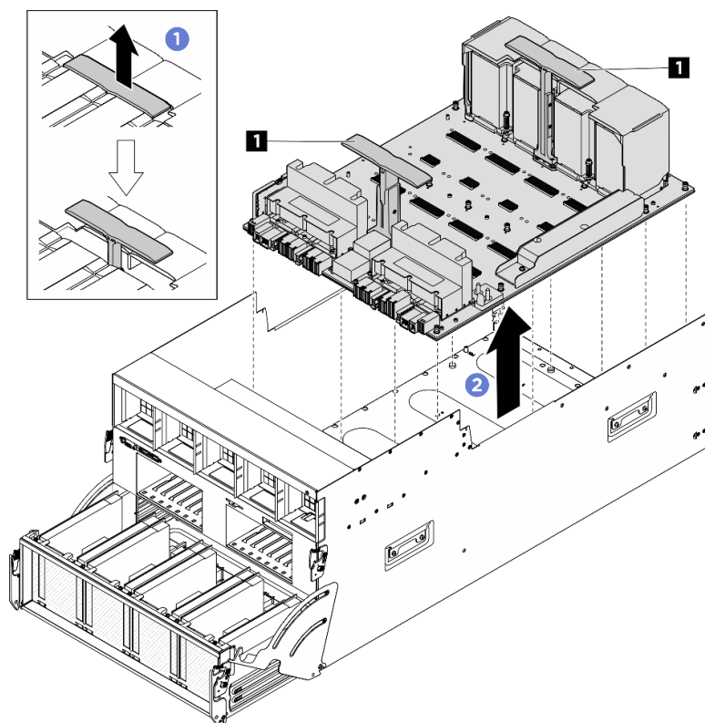
圖例 77. 卸下 GPU 基板
