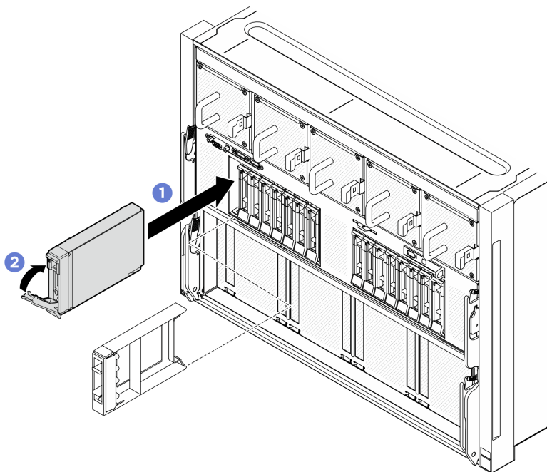
圖例 36. 安裝 2.5 吋熱抽換硬碟
