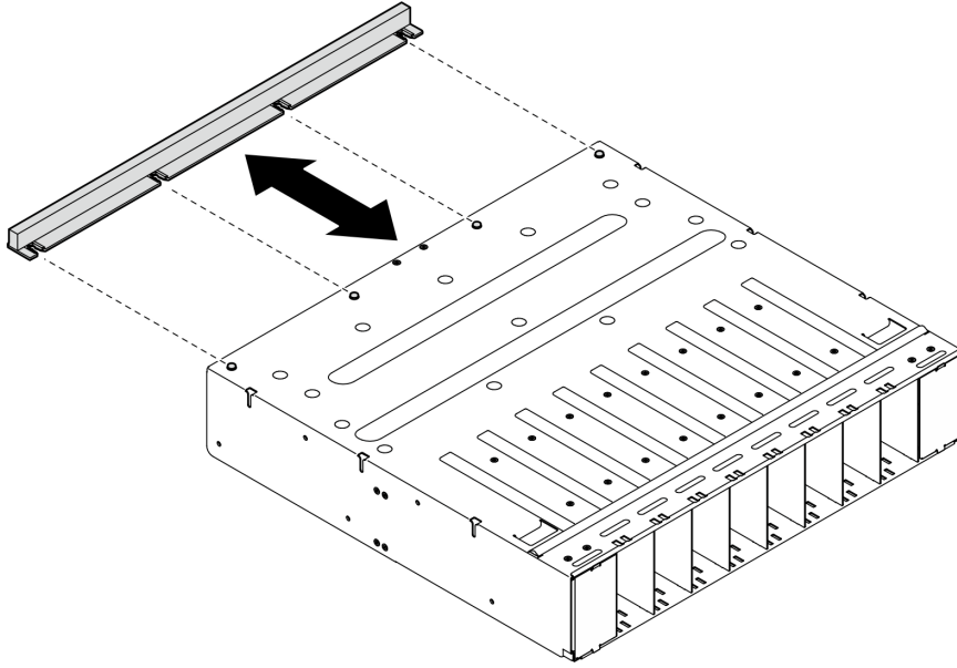
圖例 68. 安裝 GPU 空氣擋板
