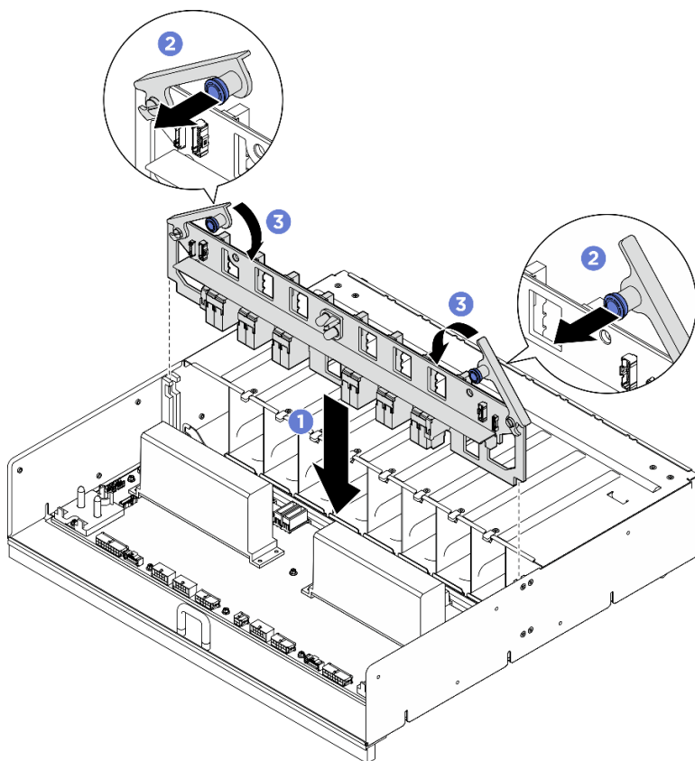
圖例 210. 安裝 PSU 轉插卡
