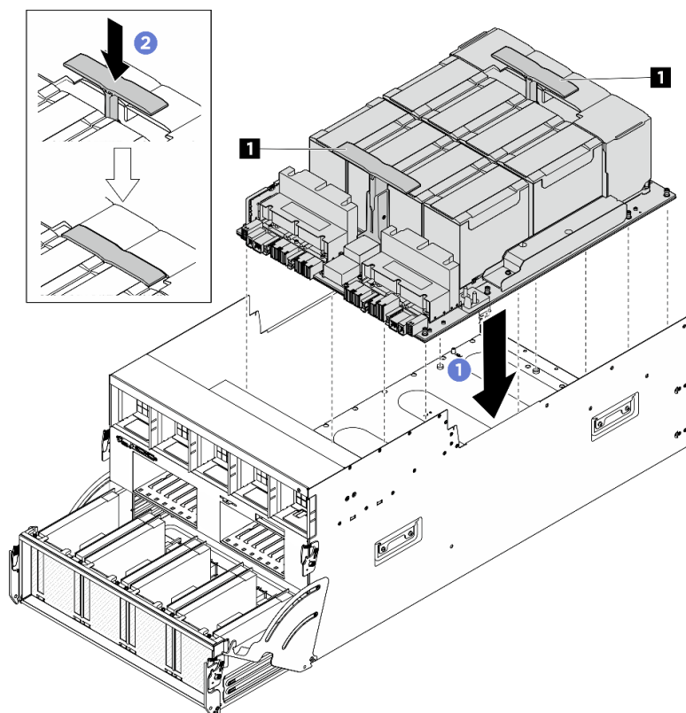
圖例 90. 安裝 GPU 複合體
