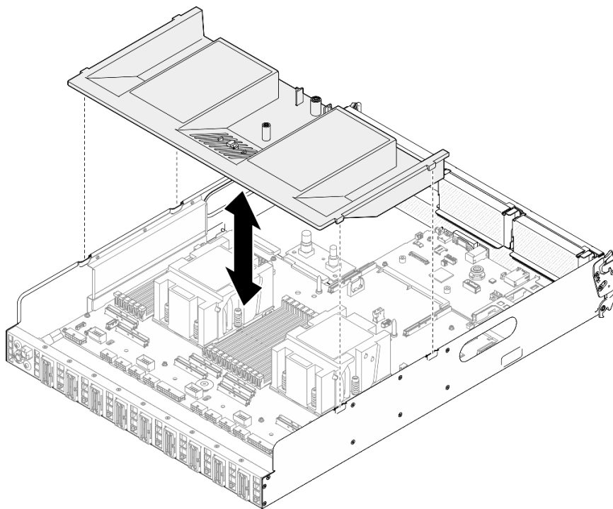
圖例 197. 安裝處理器空氣擋板
