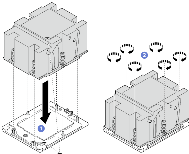
圖例 204. 安裝散熱槽
