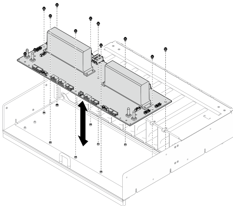
圖例 208. 安裝電源配送板
