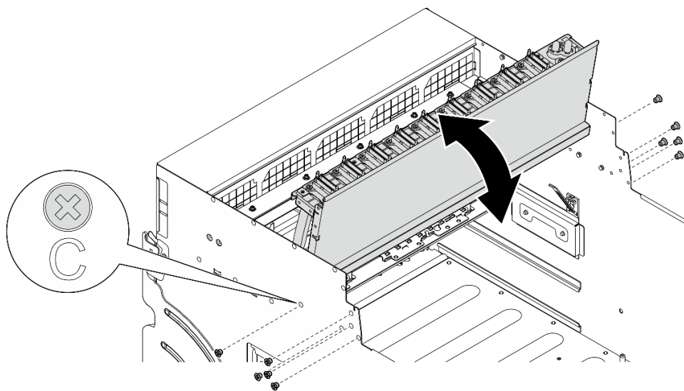
圖例 106. 翻轉前方 PCIe 交換器纜線載具
