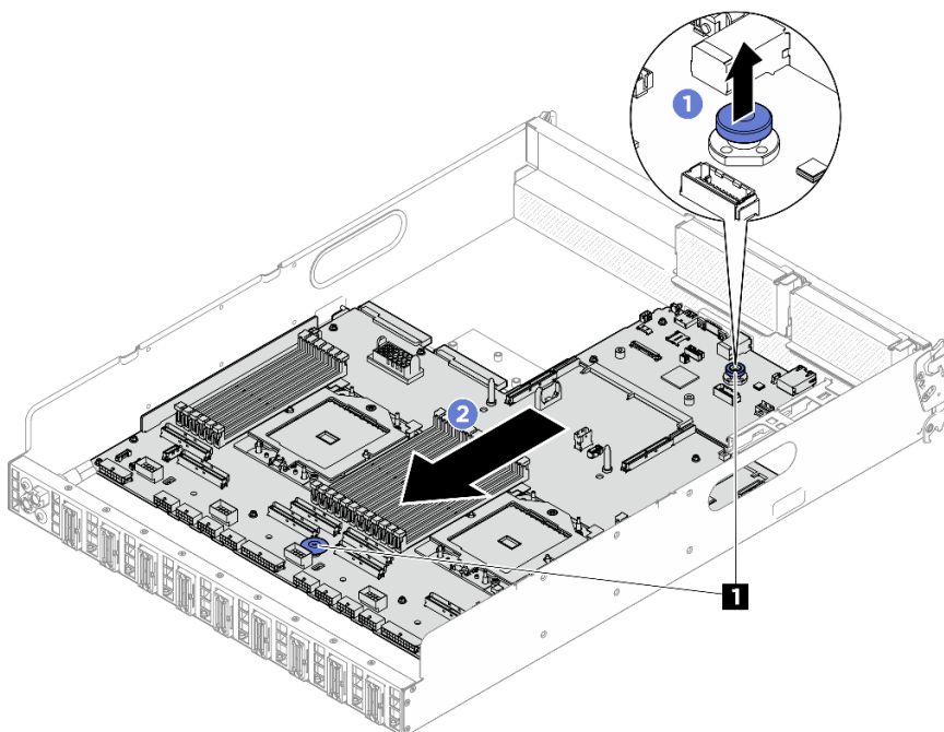
圖例 217. 鬆開主機板組件
