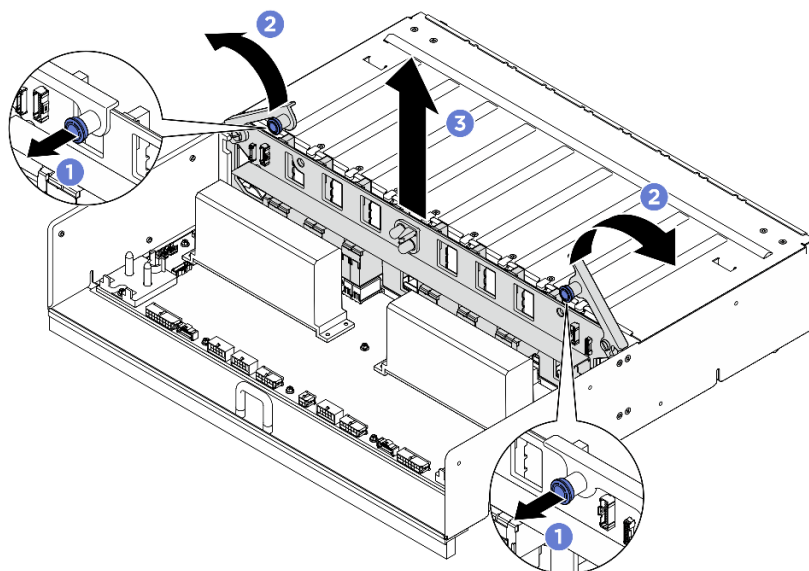
圖例 205. 卸下 PSU 轉插卡
