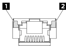
圖例 268. XCC 系統管理埠 (10/100/1000 Mbps RJ-45) LED
