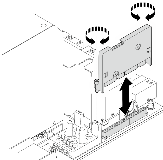
圖例 119. 卸下 HMC 卡
