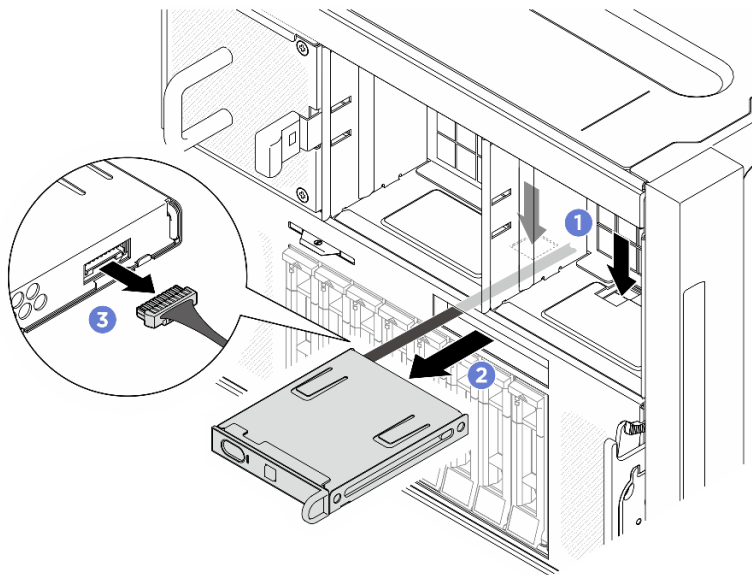
圖例 121. 卸下整合式診斷面板
