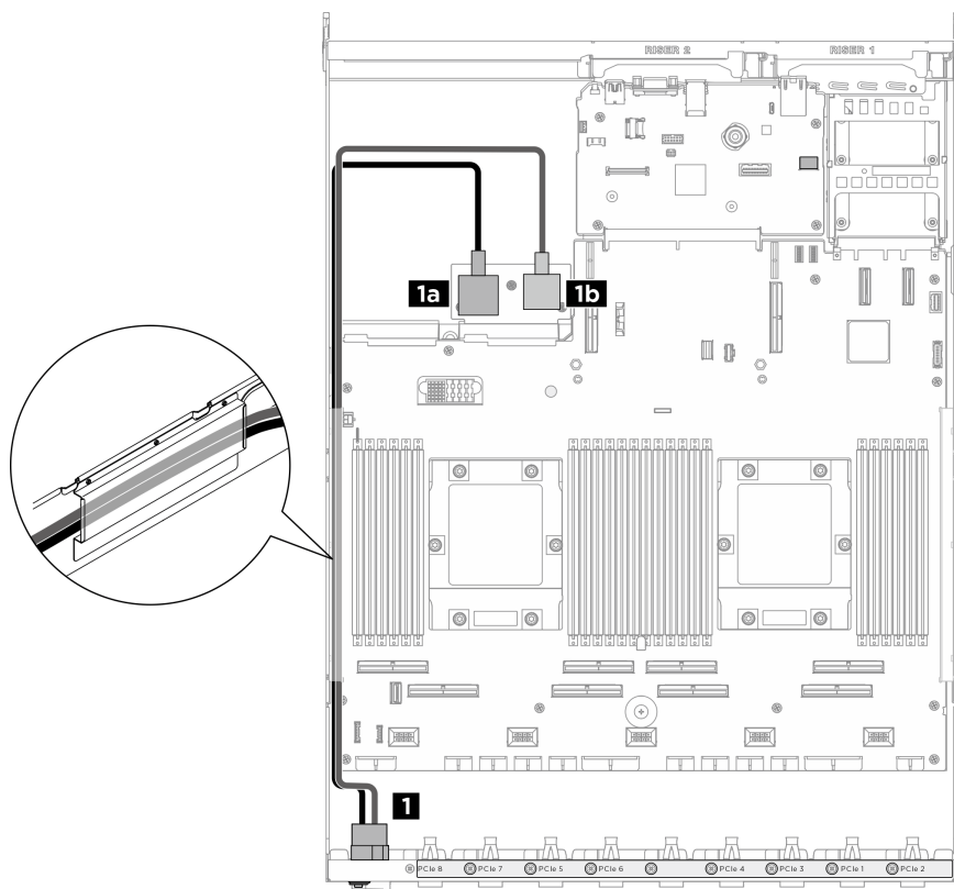
圖例 260. 電源介面板纜線佈線
