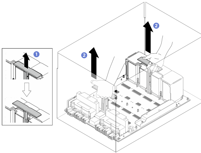
圖例 78. 從包裝盒中取出 GPU 基板
