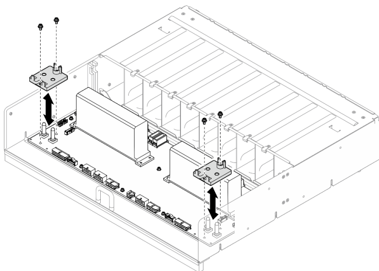
圖例 186. 卸下纜線固定器
