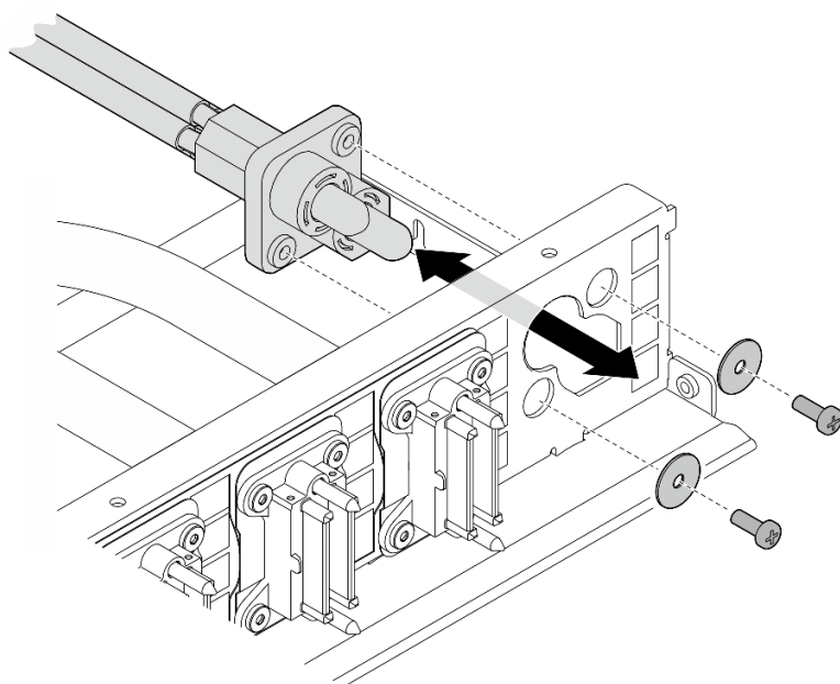
圖例 170. 安裝電源線
