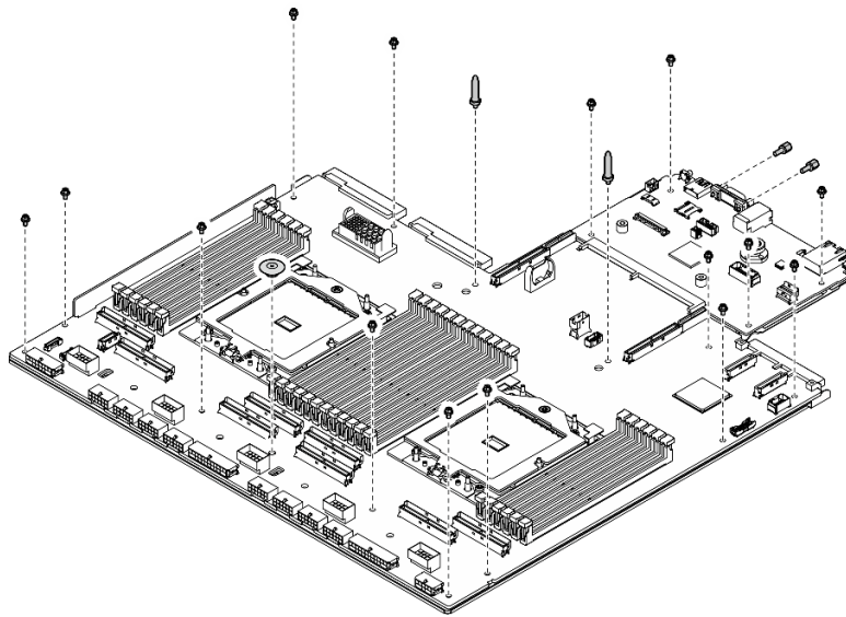
圖例 227. 安裝元件
