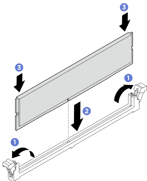
圖例 137. 安裝記憶體模組
