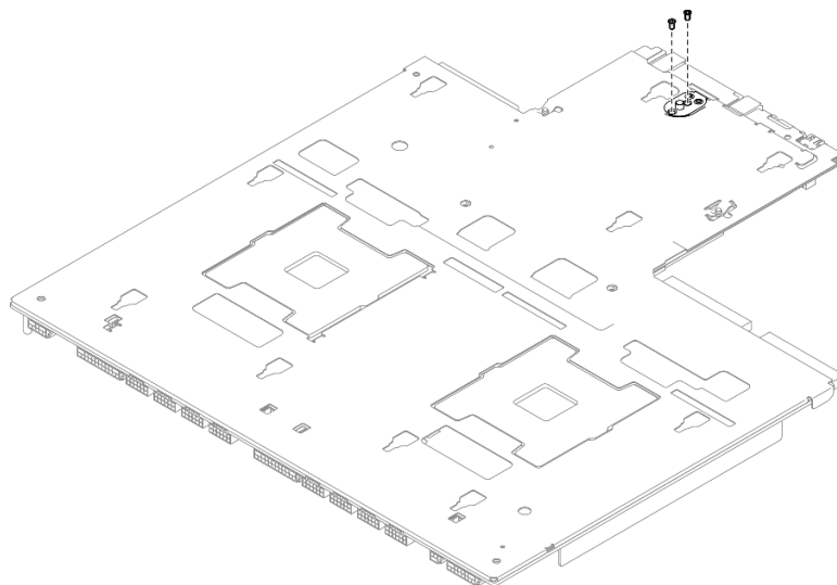
圖例 220. 卸下螺絲
