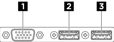
圖例 9. 正面 I/O 模組
