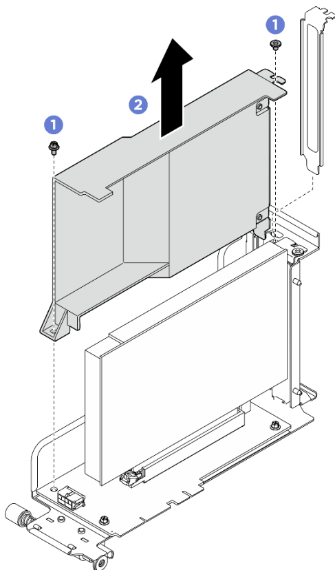
圖例 152. 卸下 PCIe 擴充卡空氣擋板
