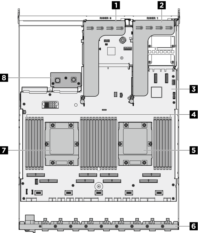
圖例 7. 2U 運算滑動箱俯視圖
