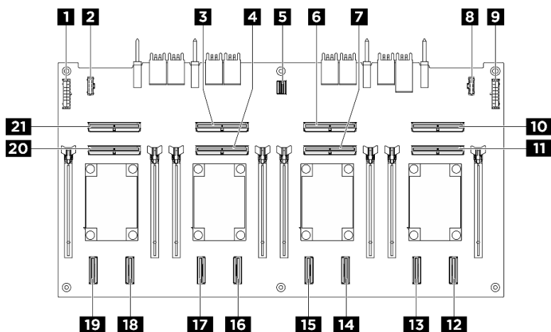
圖例 238. PCIe 交換器板接頭
