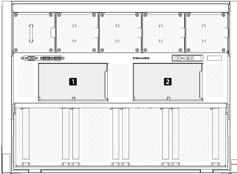
圖例 37. 2.5 吋硬碟背板編號
