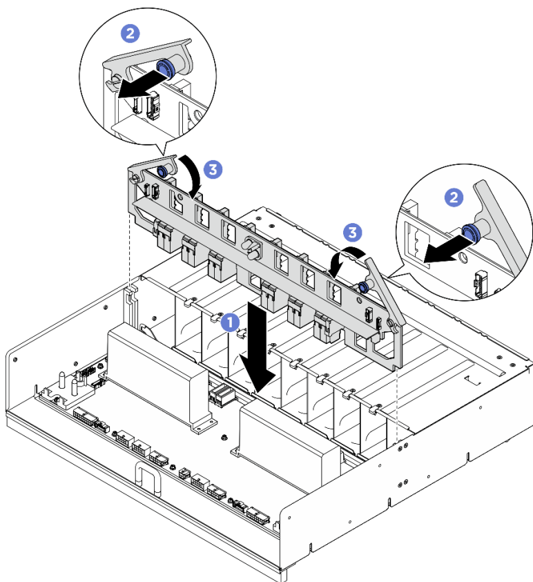
圖例 212. 安裝 PSU 轉插卡
