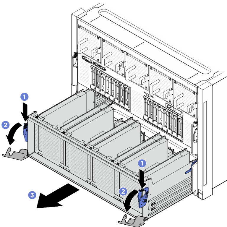
圖例 74. 將 PCIe 交換器滑動箱拉動到停止位置
