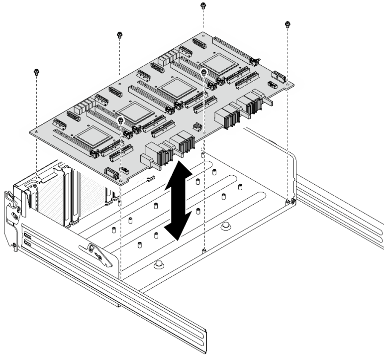
圖例 160. 安裝 PCIe 交換器板
