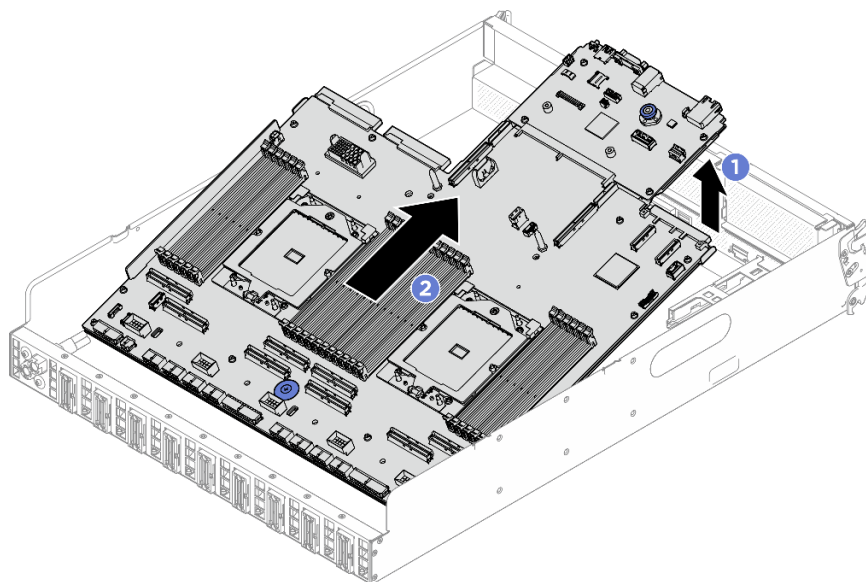
圖例 271. 卸下主機板組件
