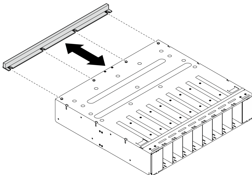
圖例 67. 卸下 GPU 空氣擋板
