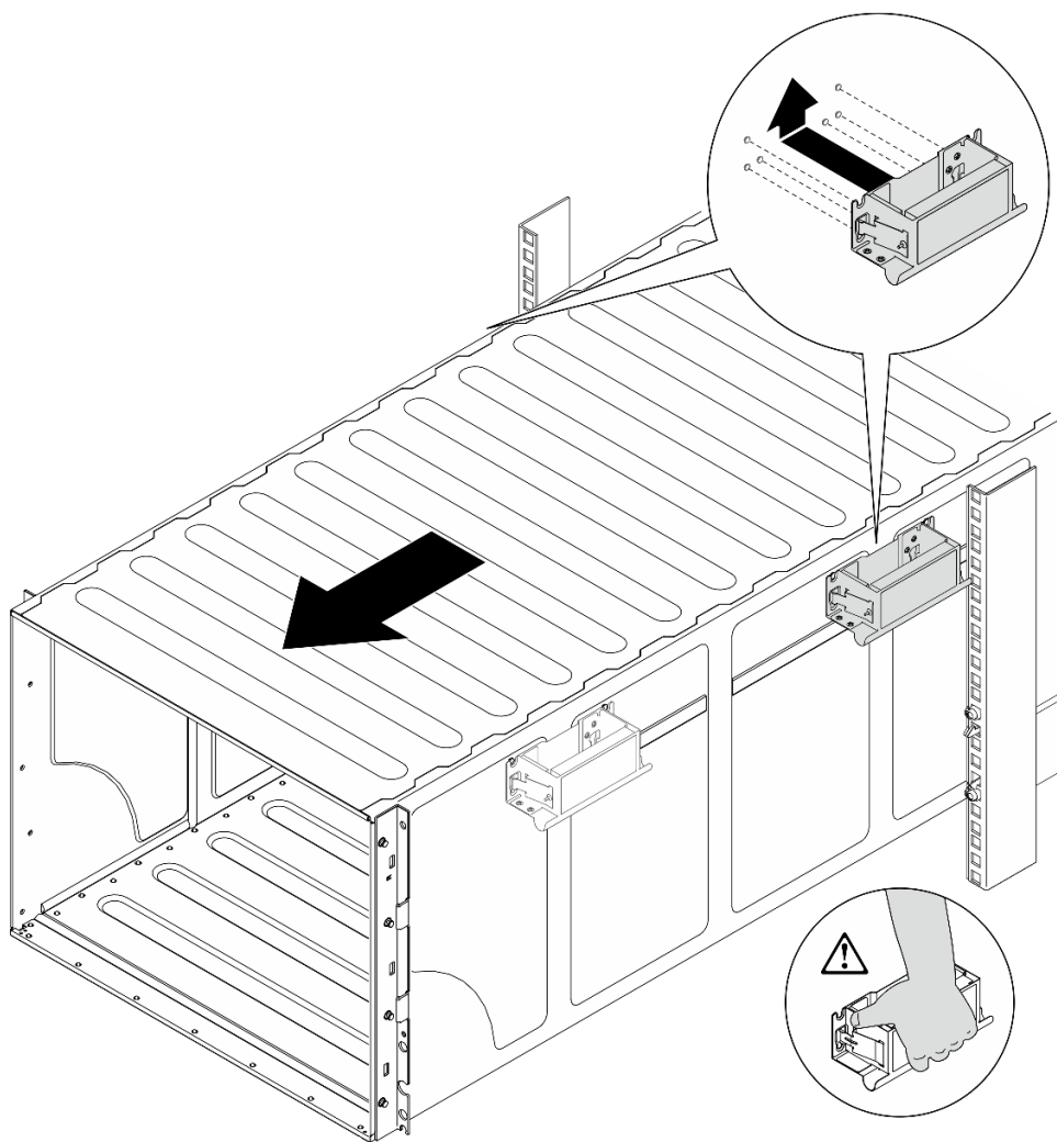
圖例 23. 安裝後把手
