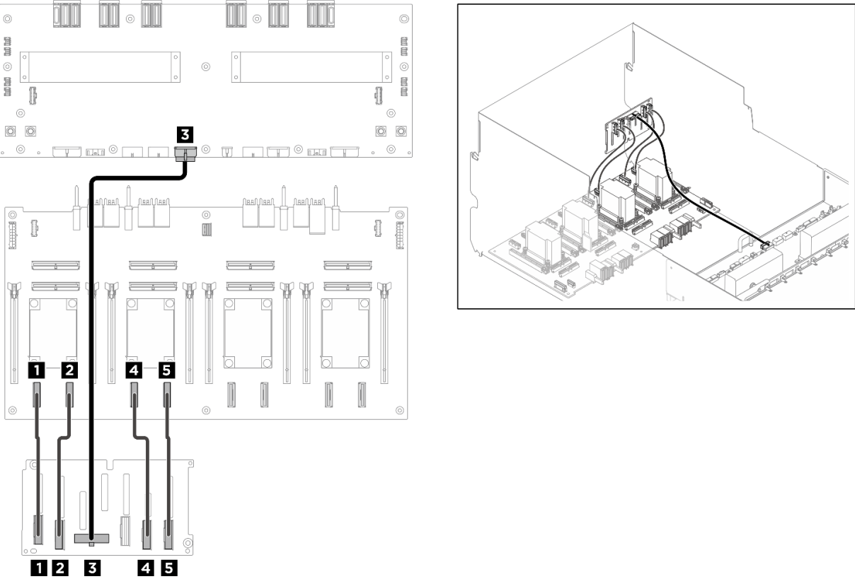
圖例 245. 背板 1 纜線佈線
