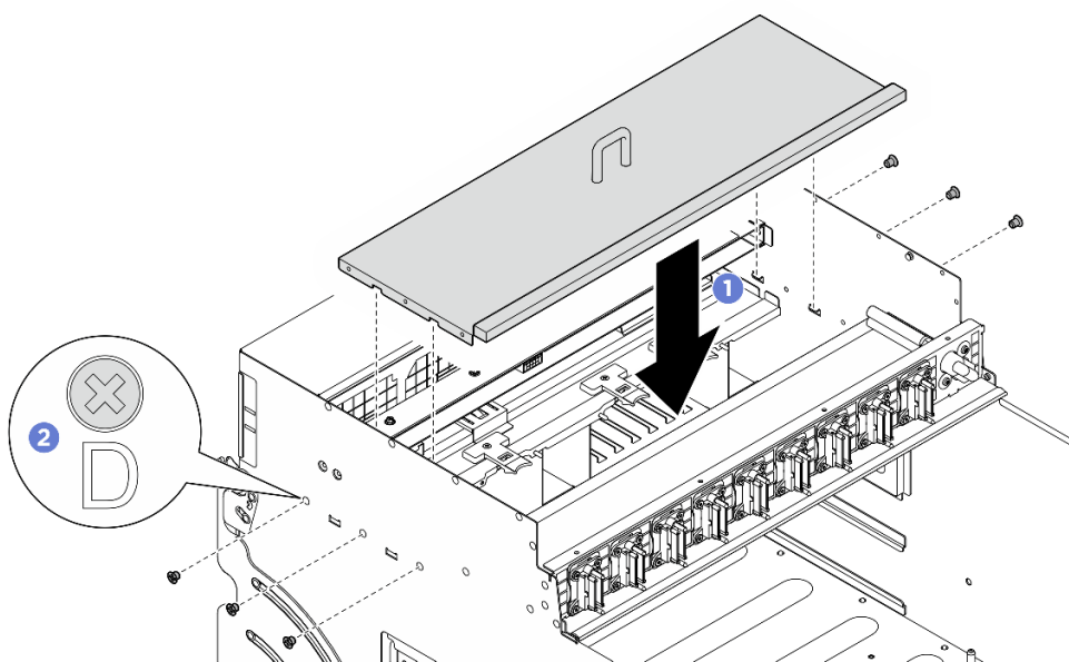
圖例 124. 安裝 I/O 蓋
