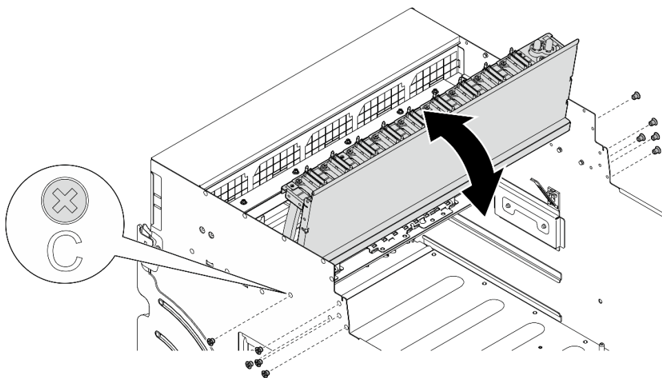
圖例 81. 翻轉前方 PCIe 交換器纜線載具
