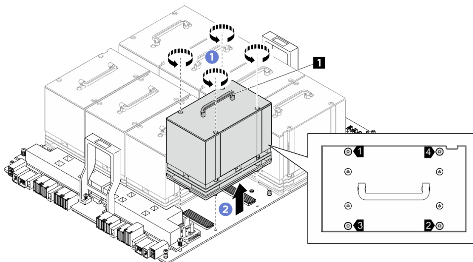
圖例 117. 卸下 GPU 和散熱槽模組
