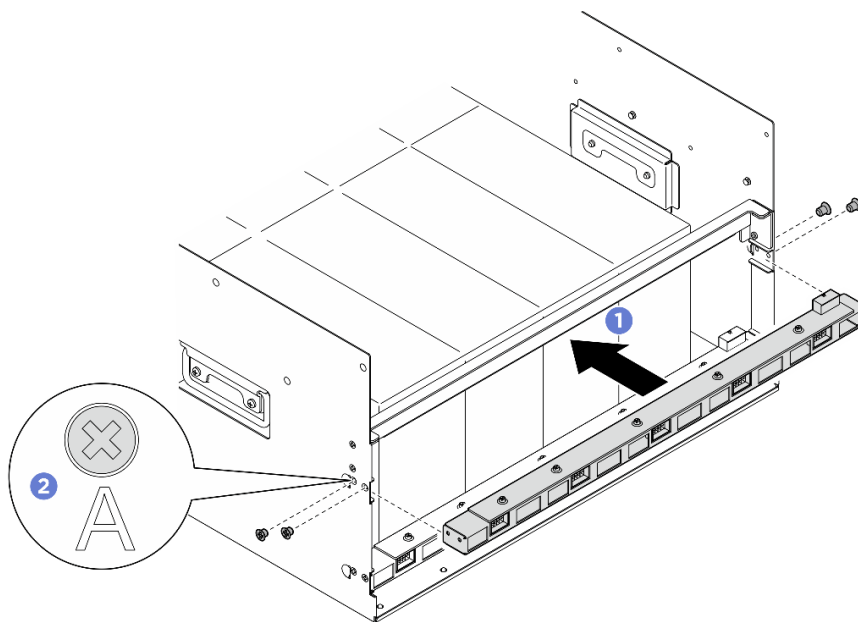
圖例 64. 安裝後方風扇控制板組件
