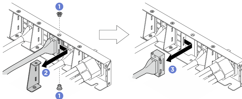
圖例 175. 卸下正面 I/O 模組、整合式診斷面板、GPU 管理或信號線
