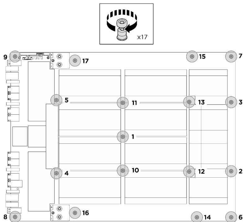
圖例 80. 安裝螺絲
