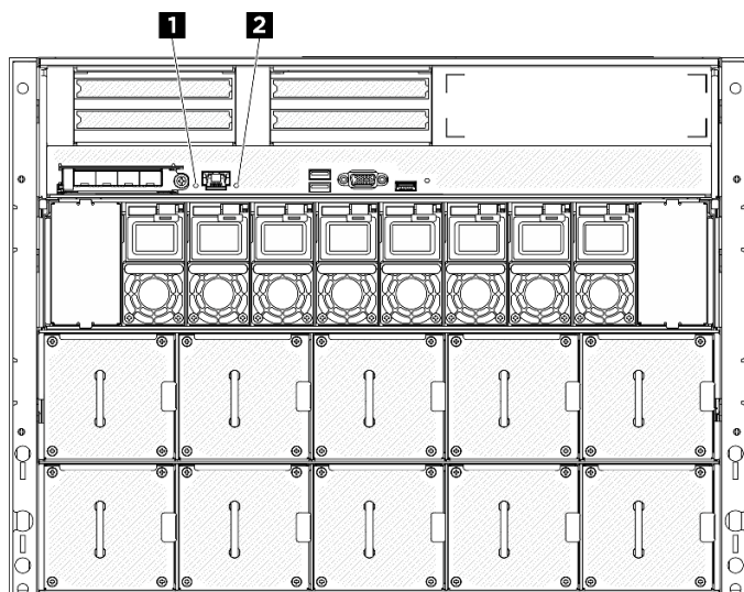
圖例 267. 背面圖上的系統 LED
