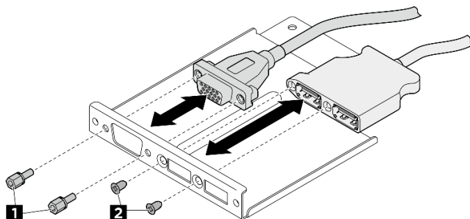
圖例 172. 安裝正面 I/O 模組纜線
