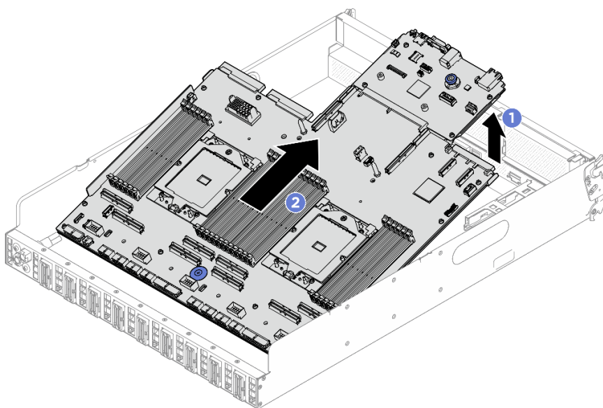
圖例 218. 卸下主機板組件
