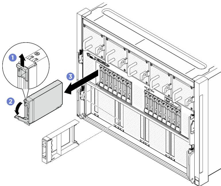
圖例 34. 卸下 2.5 吋熱抽換硬碟
