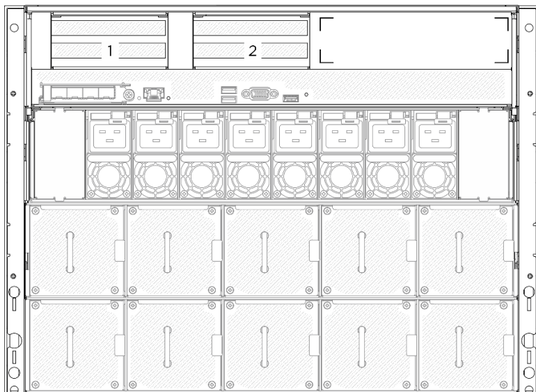
圖例 156. PCIe 擴充卡位置
