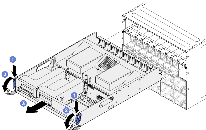
圖例 42. 卸下 2U 運算滑動箱
