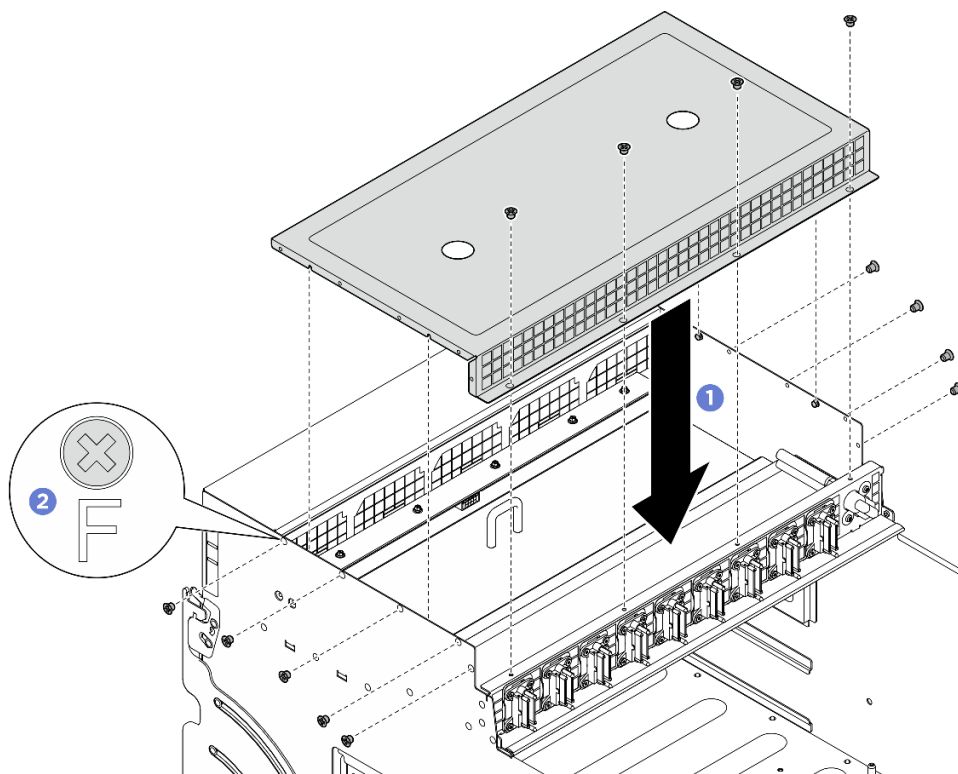
圖例 47. 安裝纜線蓋
