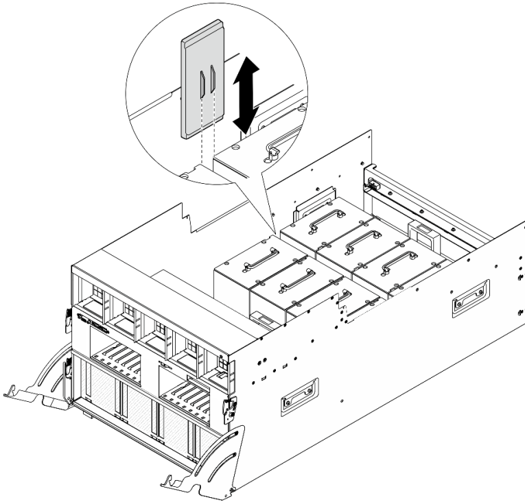
圖例 72. 安裝 GPU 空氣導管
