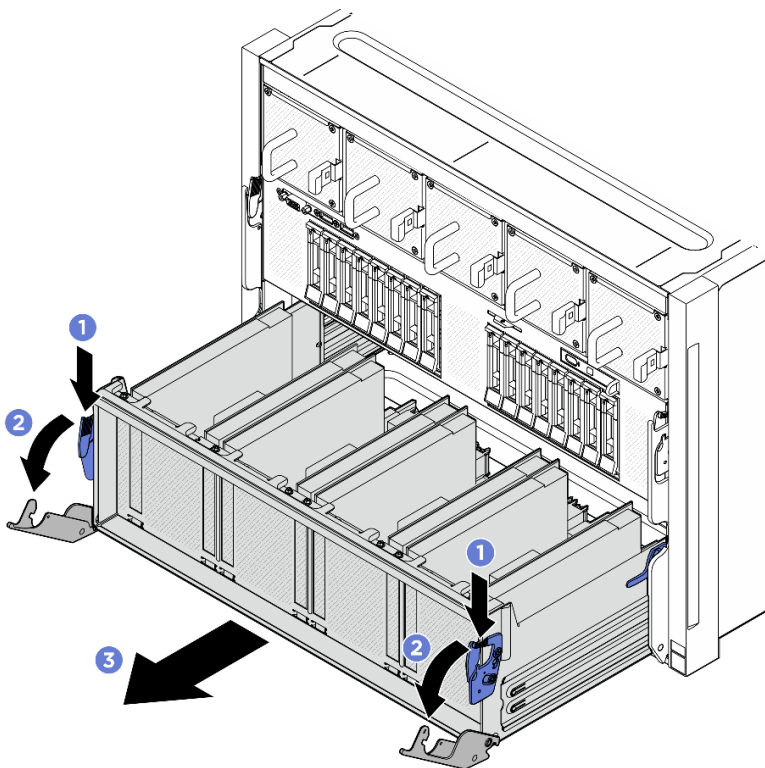
圖例 142. 將 PCIe 交換器滑動箱拉動到停止位置
