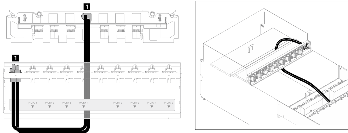
圖例 261. 電源介面板纜線佈線
