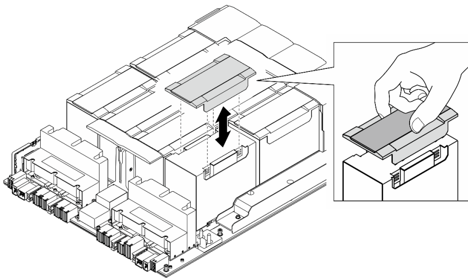
圖例 112. 卸下塑膠蓋
