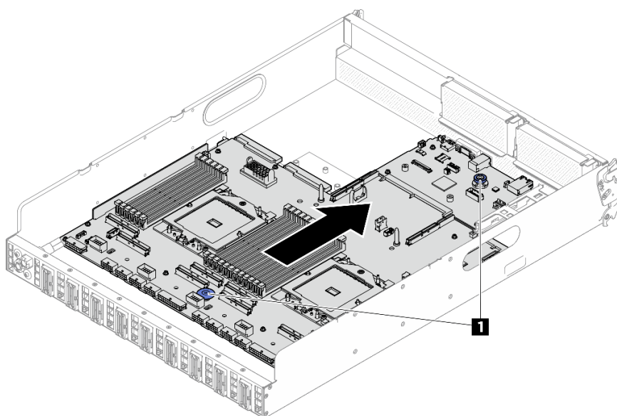
圖例 232. 安裝主機板組件
