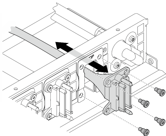
圖例 166. 卸下正面 I/O 模組、整合式診斷面板、GPU 管理或信號線
