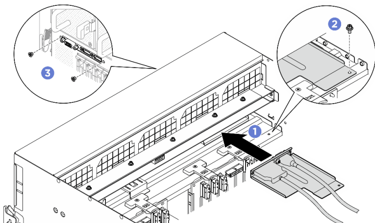
圖例 173. 安裝正面 I/O 模組
