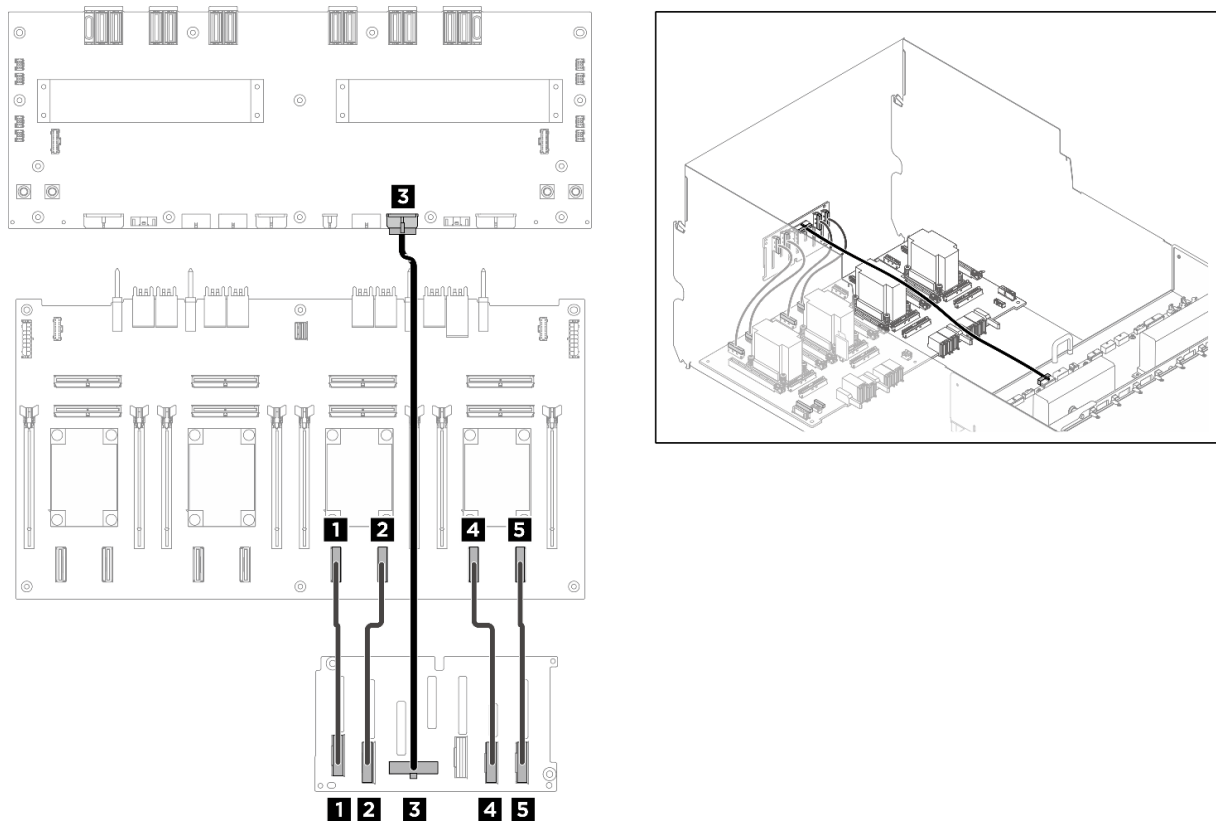
圖例 246. 背板 2 纜線佈線
