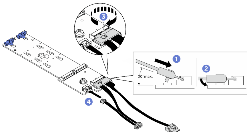
圖例 128. 連接 M.2 背板纜線
