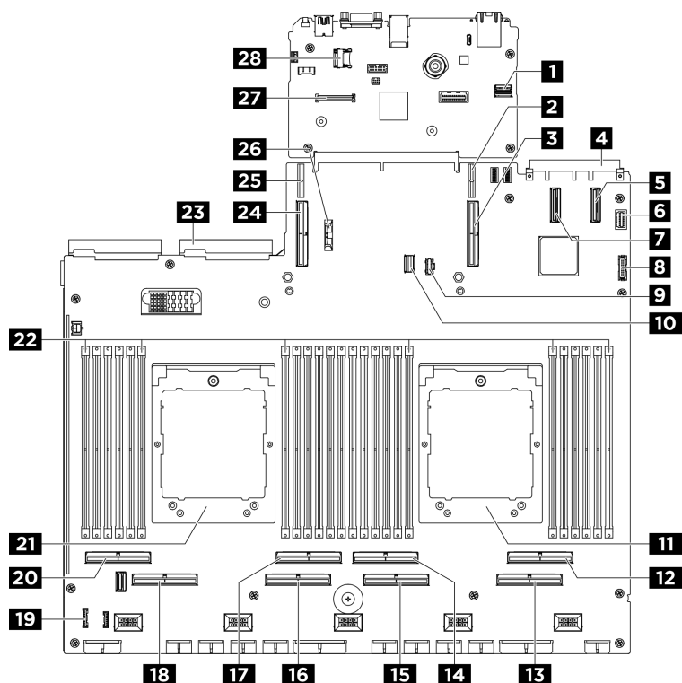
圖例 11. 主機板組件接頭
