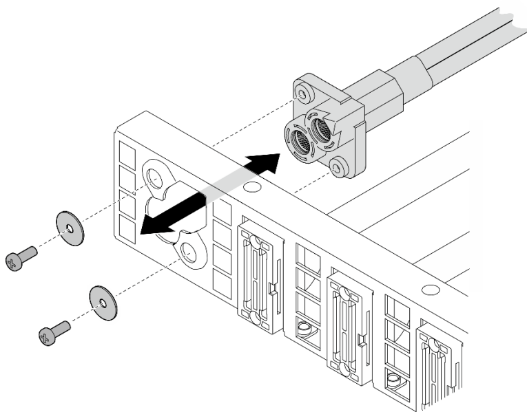
圖例 178. 安裝電源線
