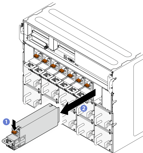
圖例 193. 電源供應器卸下
