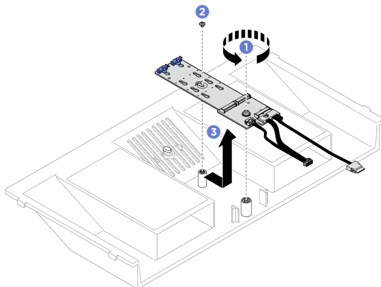
圖例 126. 卸下 M.2 背板
