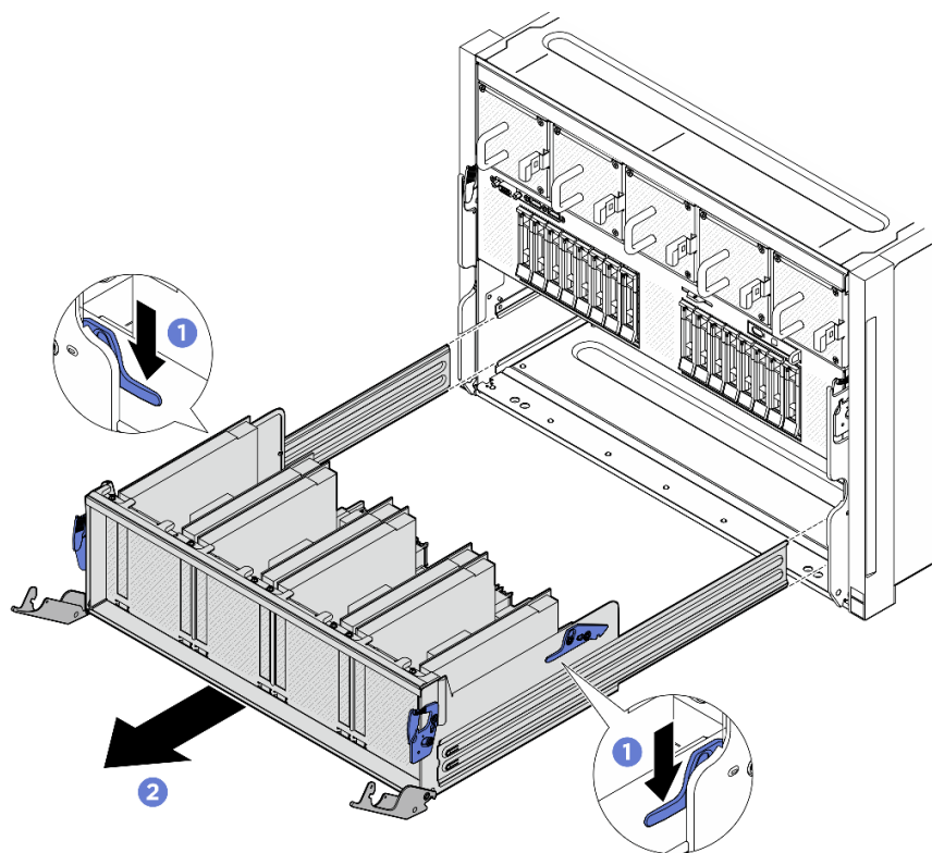
圖例 181. 將 PCIe 交換器滑動箱從 8U GPU 滑動箱卸下
