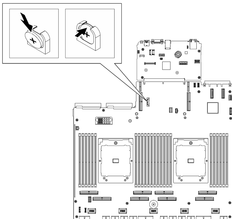
圖例 49. CMOS 電池安裝
