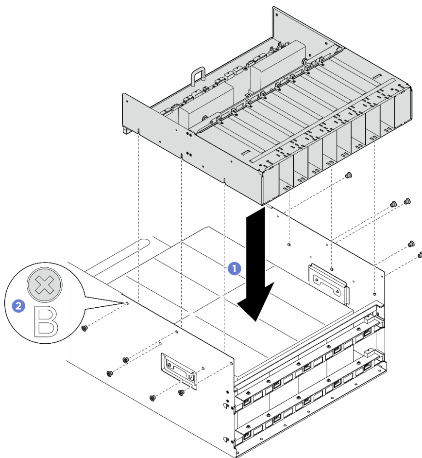
圖例 185. 安裝電源複合體
