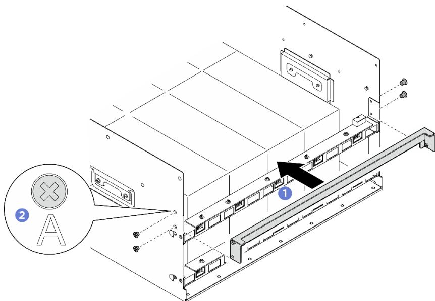
圖例 94. 安裝後支撐托架
