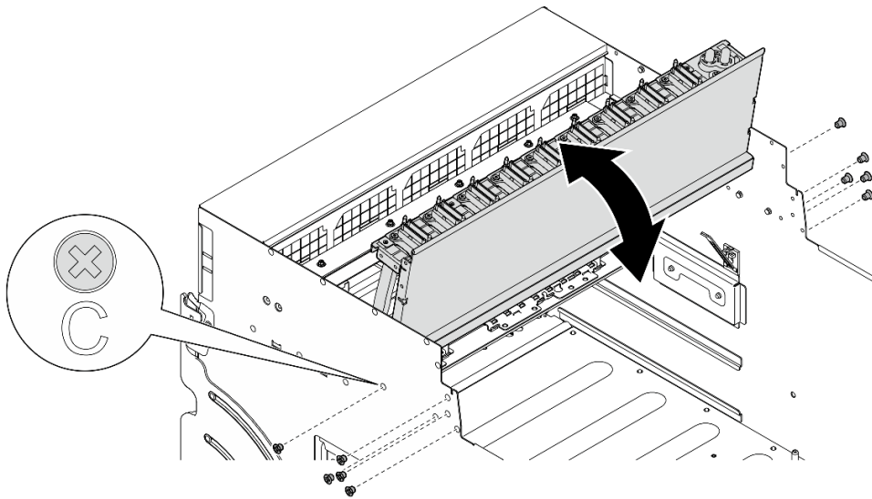
圖例 92. 翻轉前方 PCIe 交換器纜線載具
