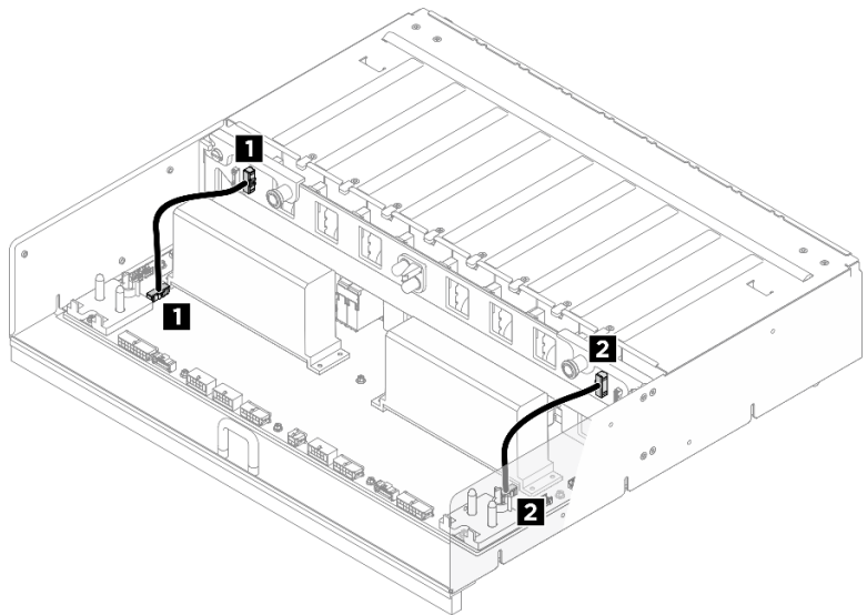
圖例 262. PSU 轉插卡纜線佈線
