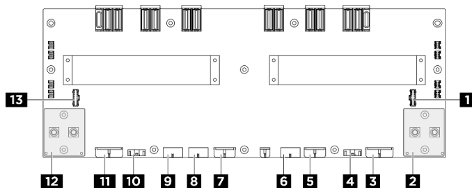
圖例 241. 電源配送板接頭
