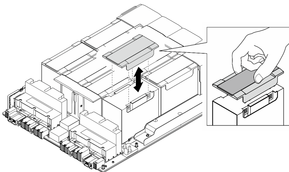
圖例 116. 安裝塑膠蓋
