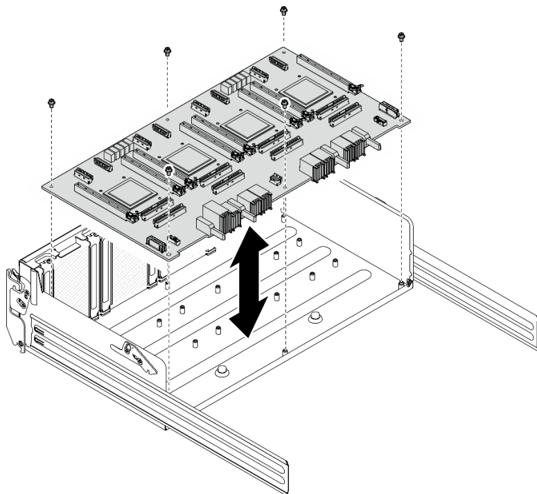
圖例 159. 卸下 PCIe 交換器板
