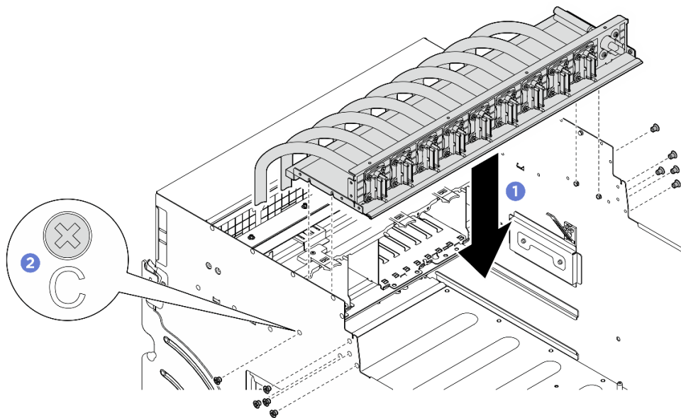
圖例 171. 安裝前方 PCIe 交換器纜線載具
