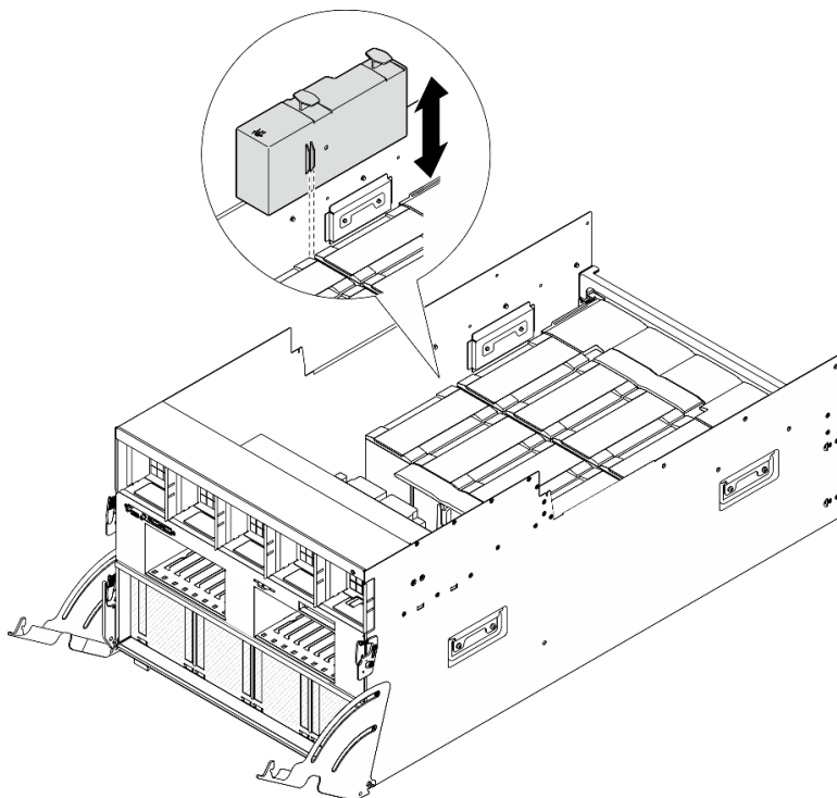
圖例 70. 安裝 GPU 空氣導管
