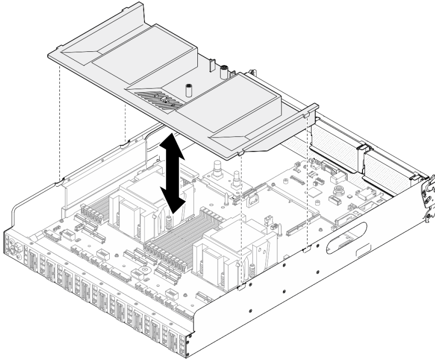
圖例 196. 卸下處理器空氣擋板
