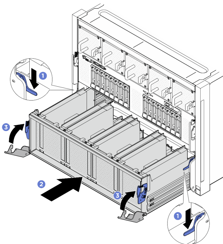
圖例 82. 將 PCIe 交換器滑動箱安裝到 8U GPU 滑動箱中
