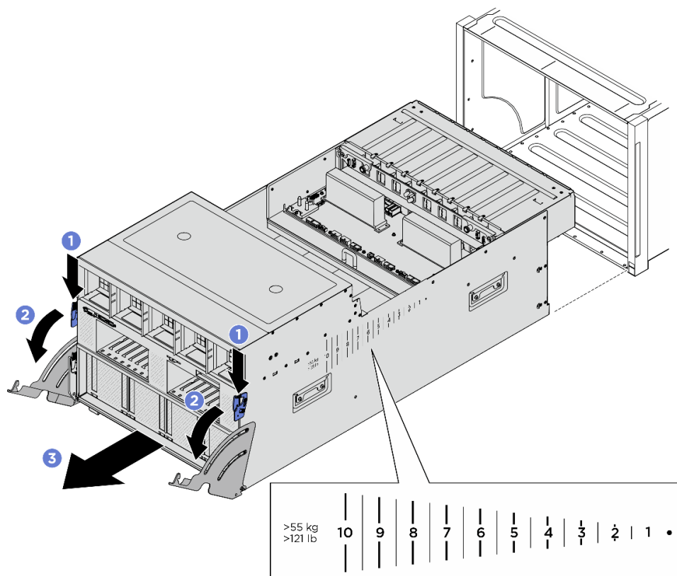
圖例 44. 卸下 8U GPU 滑動箱
