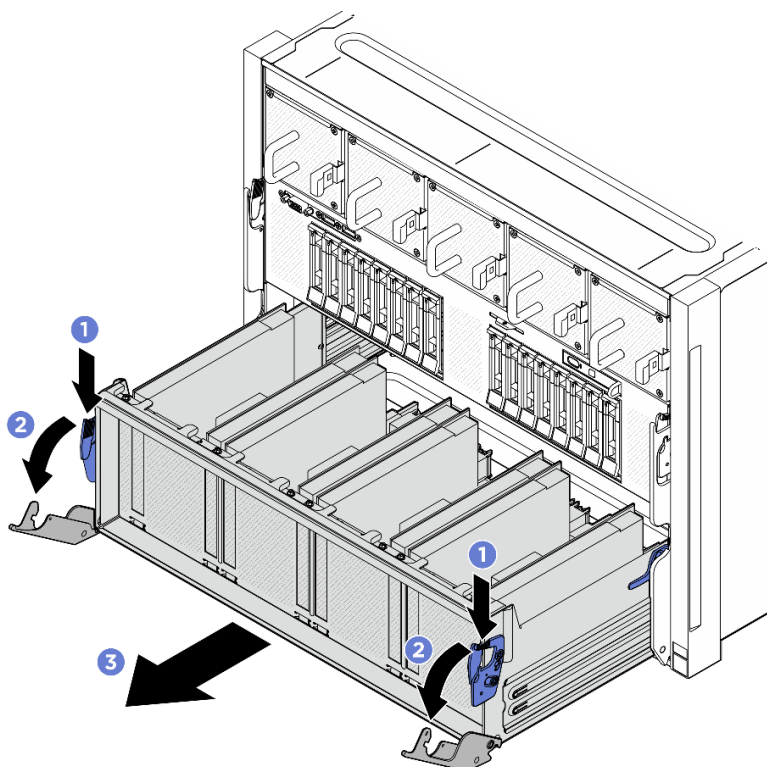
圖例 180. 將 PCIe 交換器滑動箱拉動到停止位置
