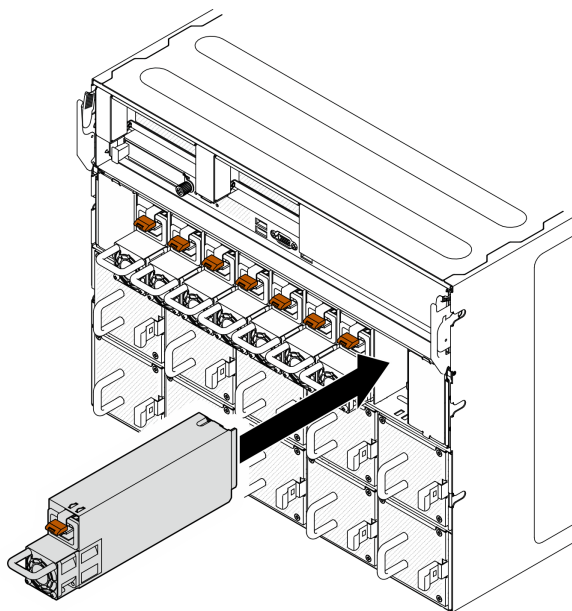
圖例 195. 安裝電源供應器
