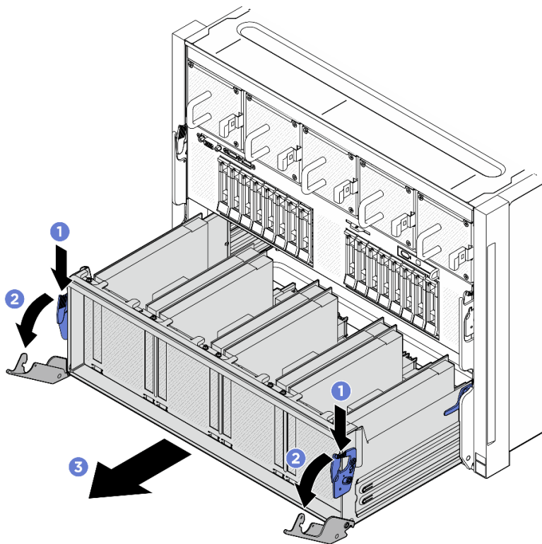
圖例 96. 將 PCIe 交換器滑動箱拉動到停止位置
