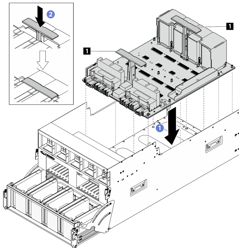
圖例 79. 安裝 GPU 基板
