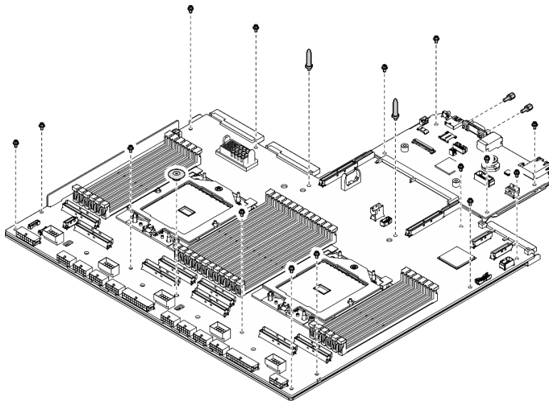
圖例 275. 卸下元件
