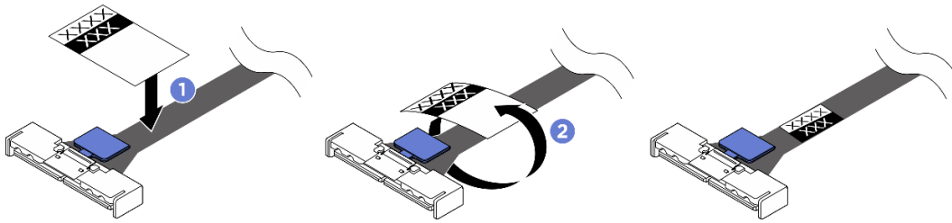
圖例 168. 黏貼標籤
