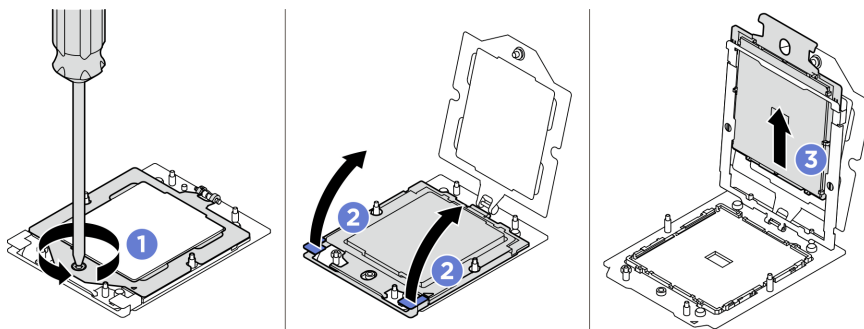
圖例 201. 卸下處理器
