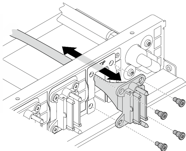
圖例 169. 安裝正面 I/O 模組、整合式診斷面板、GPU 管理或信號線
