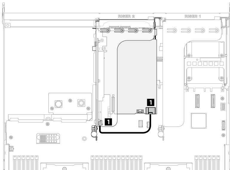
圖例 248. DPU 配接卡纜線佈線
