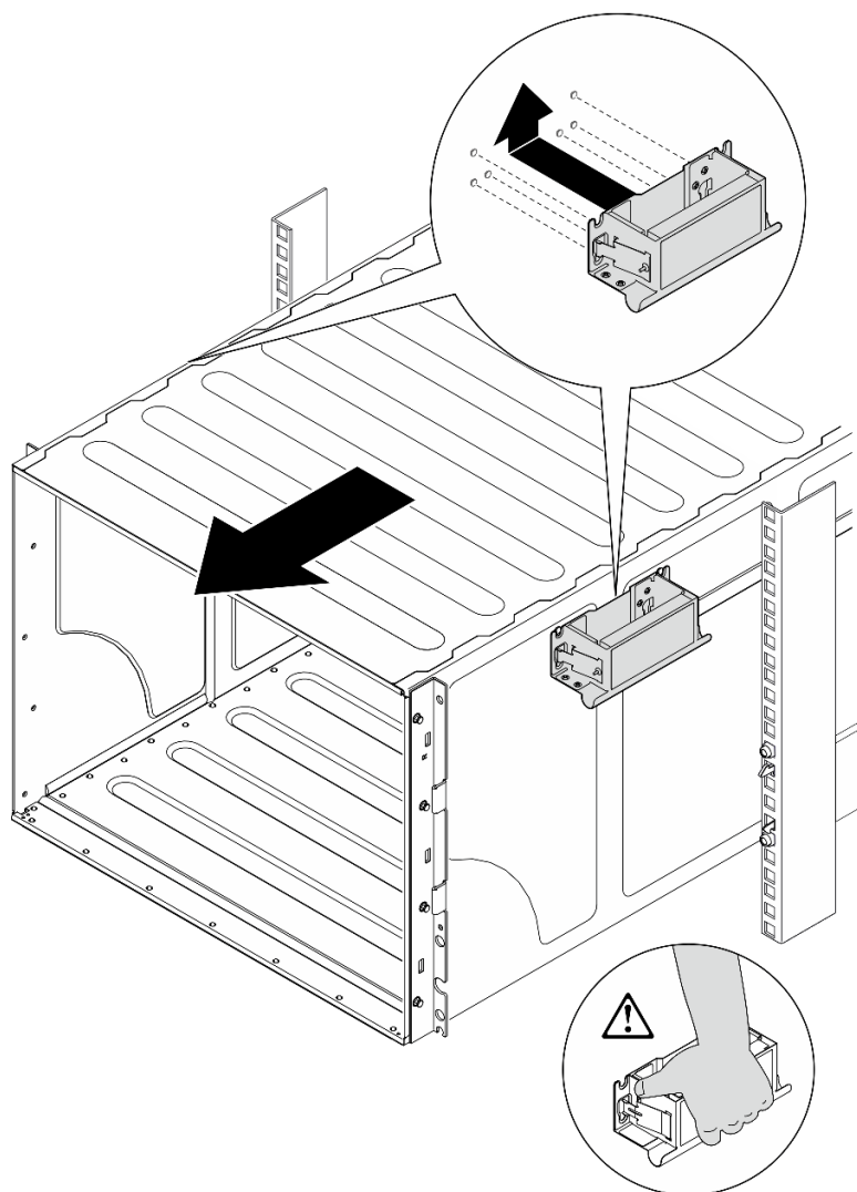
圖例 22. 安裝前把手
