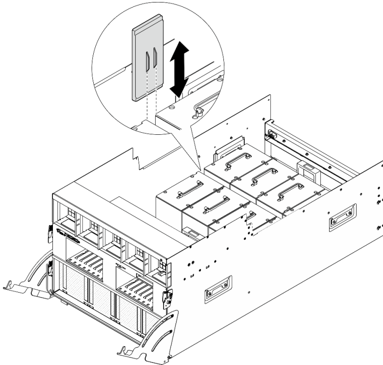
圖例 71. 卸下 GPU 空氣導管
