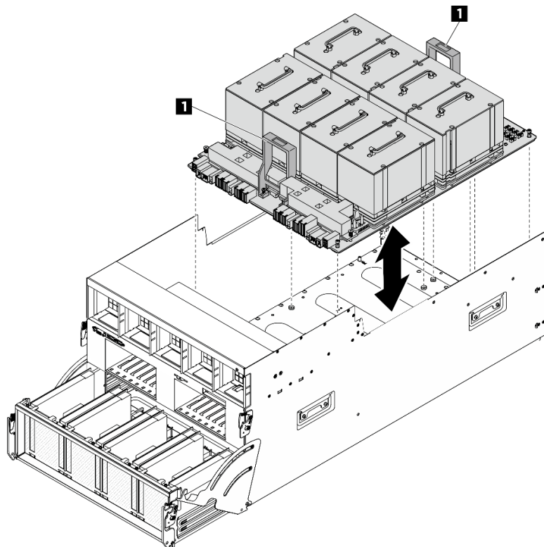
圖例 99. 卸下 GPU 複合體
