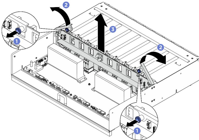
圖例 211. 卸下 PSU 轉插卡
