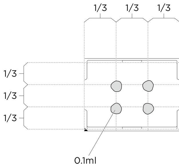
圖例 203. 塗上散熱膏
