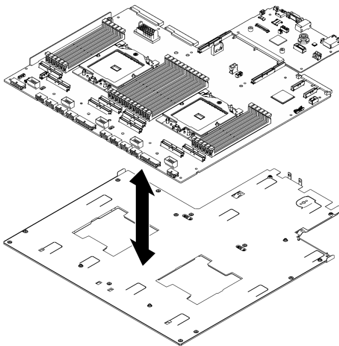
圖例 276. 拆卸主機板組件
