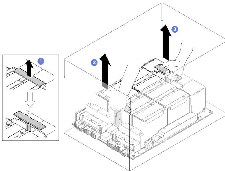
圖例 89. 從包裝盒中取出 GPU 複合體
