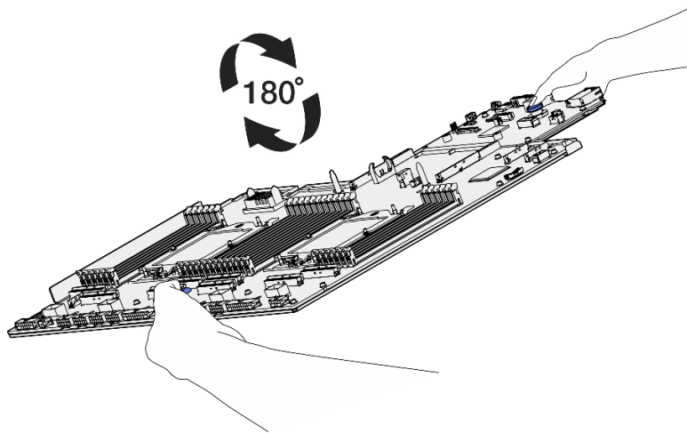
圖例 228. 將主機板組件上下倒置
