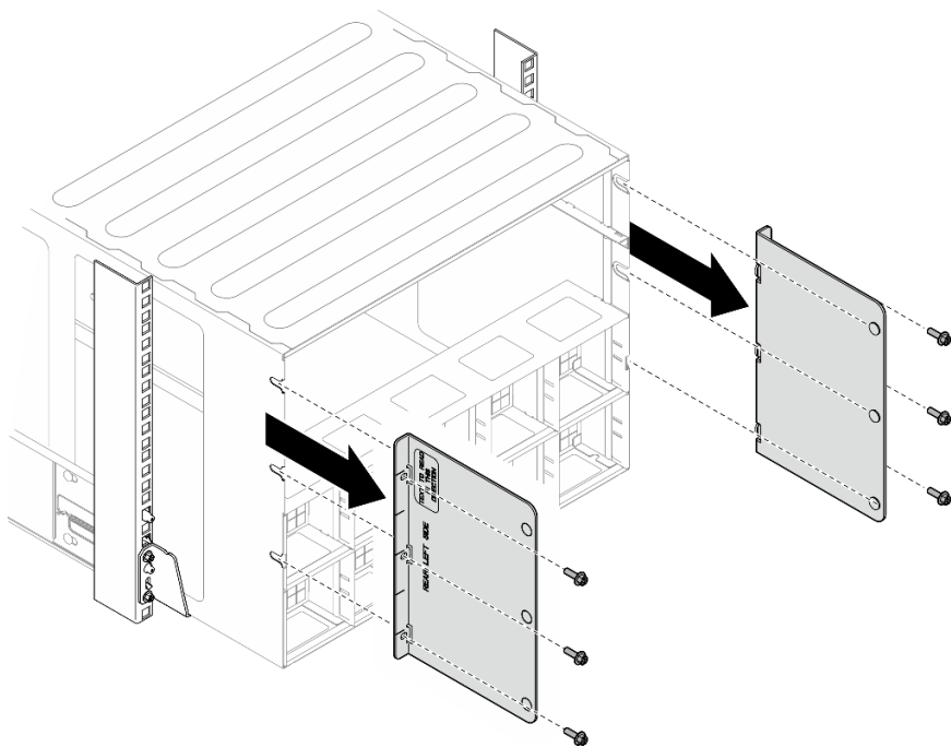
圖例 18. 卸上下支撐托架
