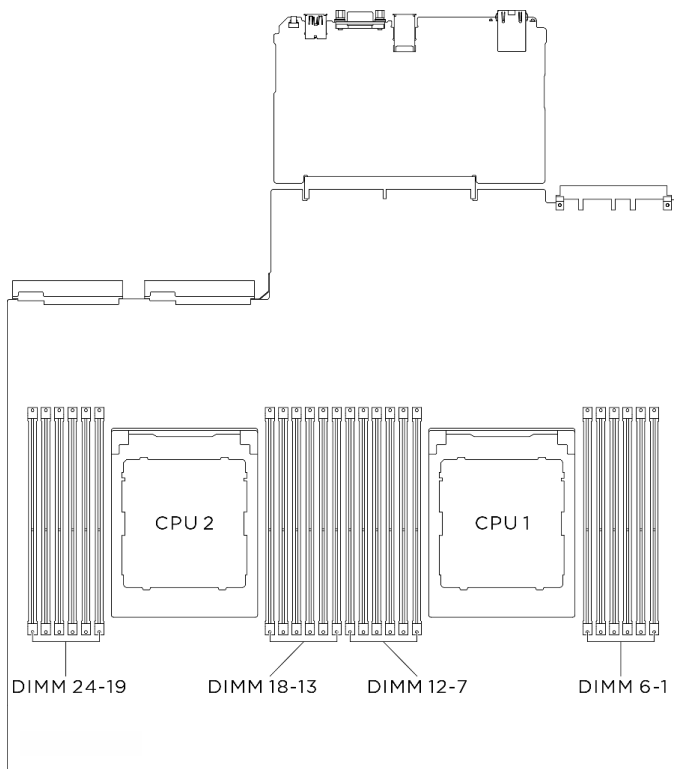
圖例 17. 記憶體模組和處理器佈置
