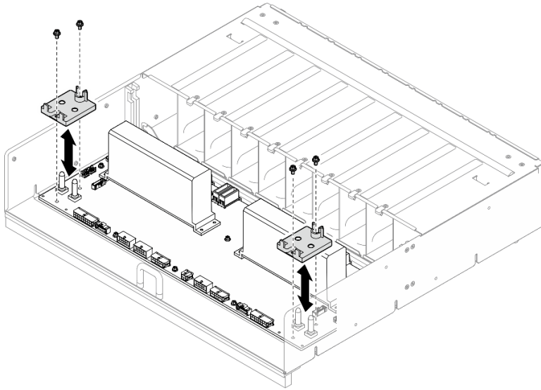
圖例 189. 安裝纜線固定器
