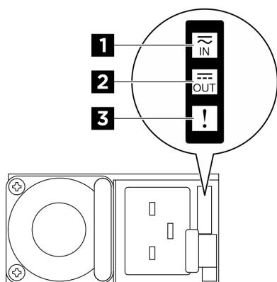
圖例 266. CFFv4 電源供應器 LED
