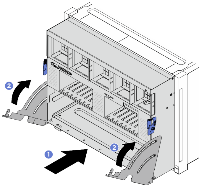
圖例 45. 安裝 8U GPU 滑動箱
