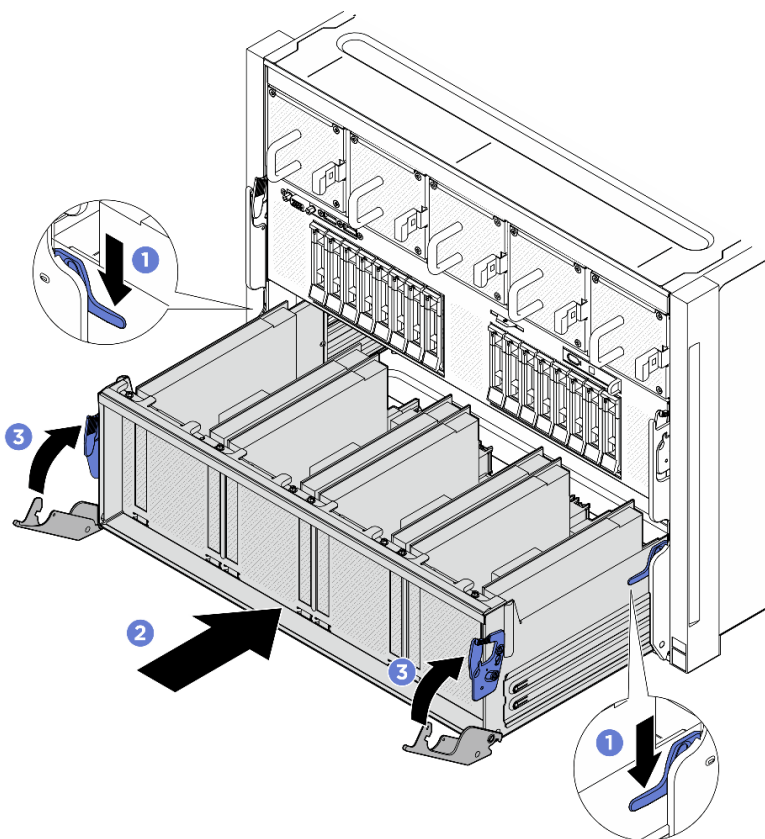
圖例 110. 將 PCIe 交換器滑動箱安裝到 8U GPU 滑動箱中
