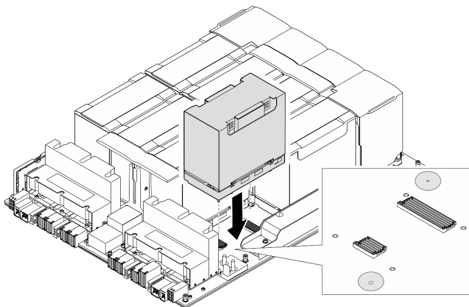
圖例 114. 安裝 GPU 和散熱槽模組
