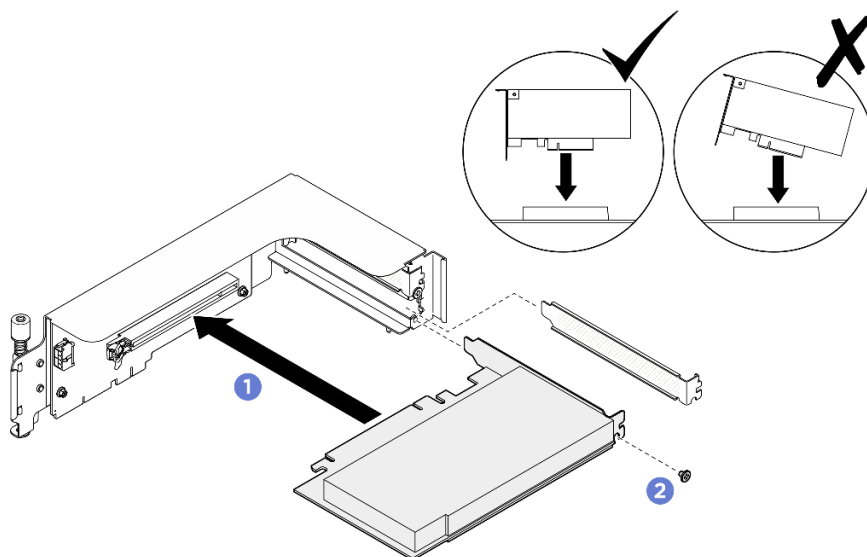
圖例 147. 安裝背面 PCIe 配接卡
