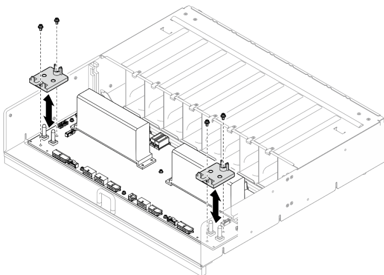
圖例 209. 安裝纜線固定器
