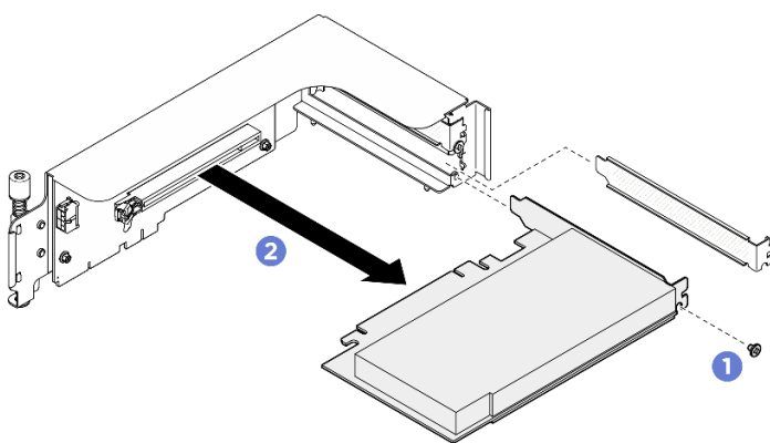
圖例 153. 卸下背面 PCIe 配接卡
