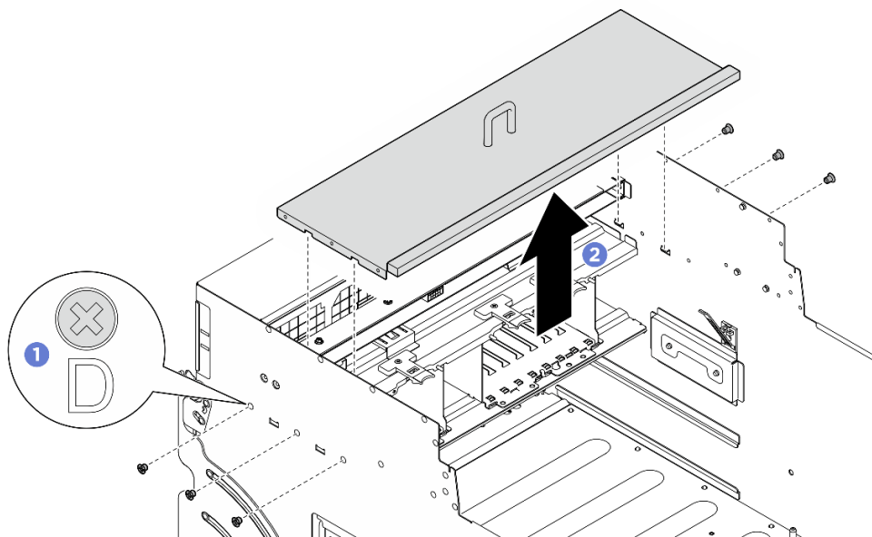
圖例 123. 卸下 I/O 蓋
