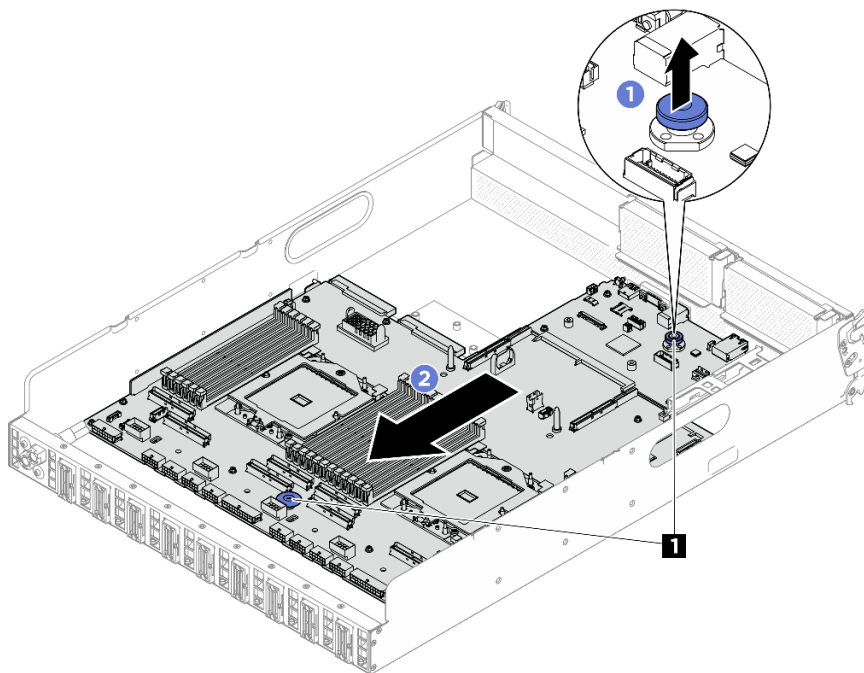
圖例 270. 鬆開主機板組件
