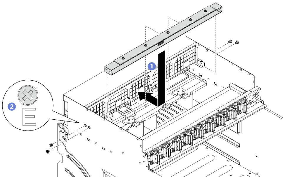
圖例 59. 安裝前方風扇控制板組件
