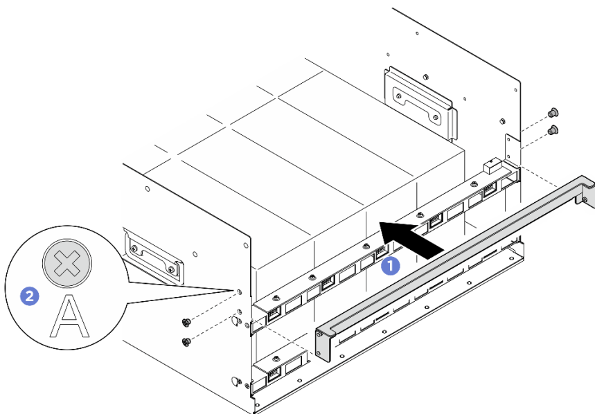
圖例 83. 安裝後支撐托架
