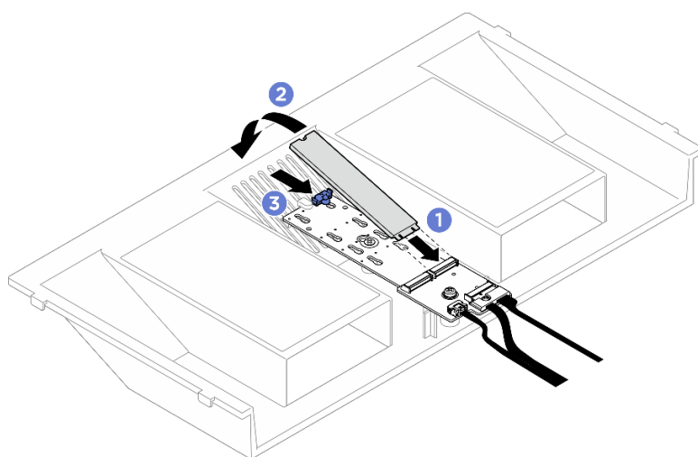
圖例 133. M.2 硬碟安裝
