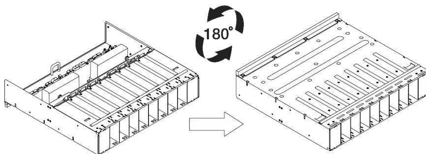
圖例 66. 將電源複合體上下倒置
