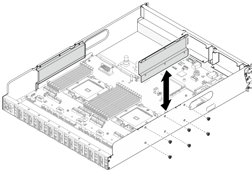
圖例 269. 卸下纜線導件
