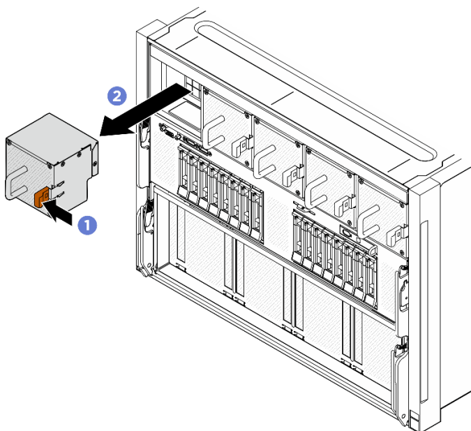
圖例 52. 熱抽換風扇卸下
