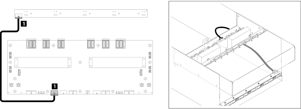
圖例 251. 後方風扇控制板（下）纜線佈線
