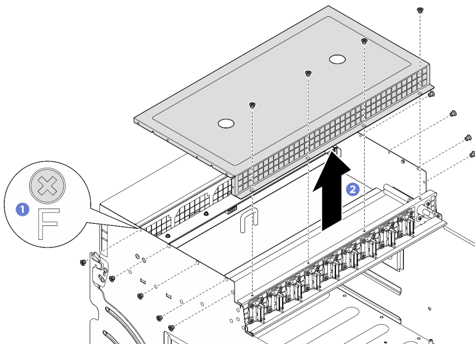
圖例 46. 卸下纜線蓋
