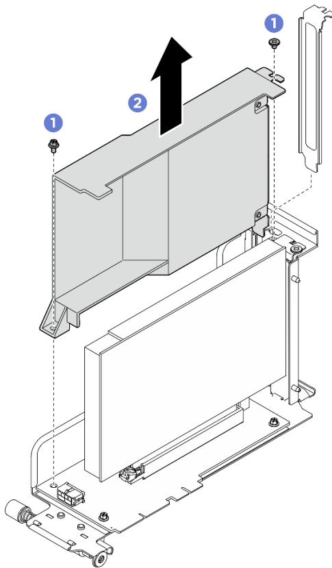
圖例 148. 卸下 PCIe 擴充卡空氣擋板
