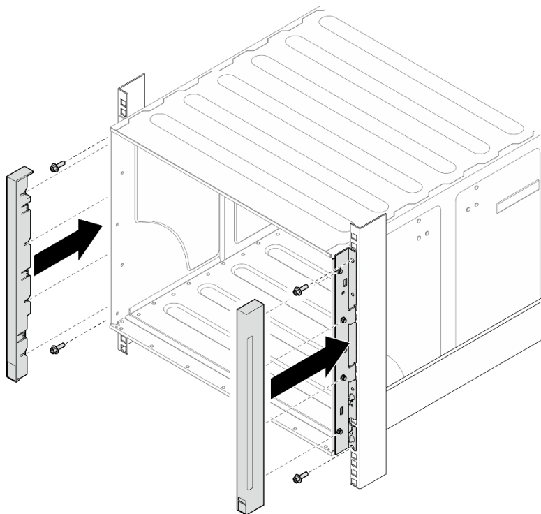
圖例 30. 安裝 EIA 蓋板
