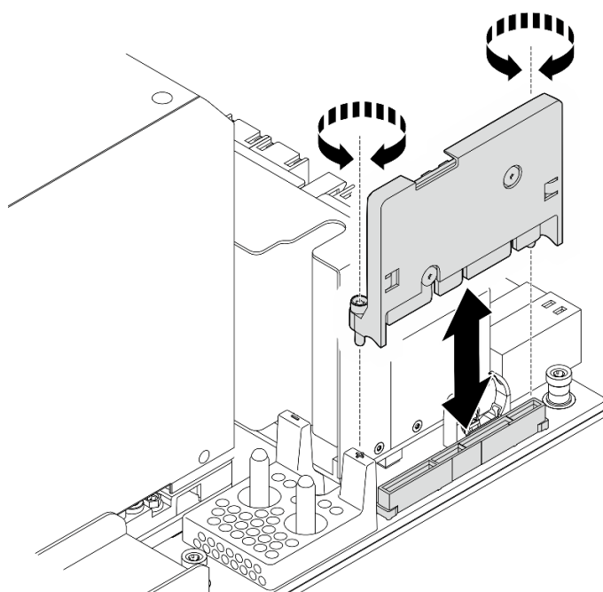
圖例 120. 安裝 HMC 卡
