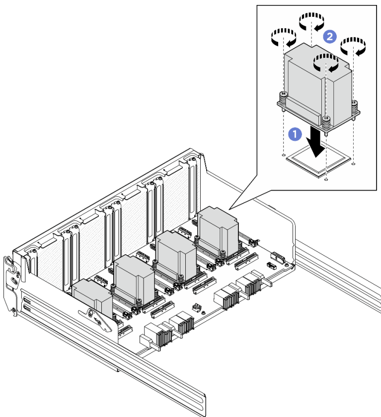
圖例 162. 安裝 PCIe 交換器板散熱槽
