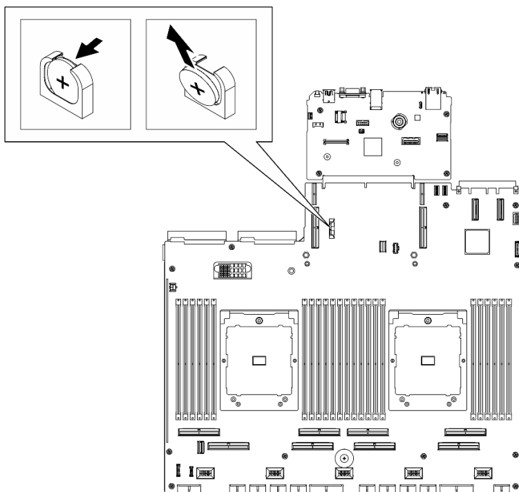
圖例 48. 卸下 CMOS 電池
