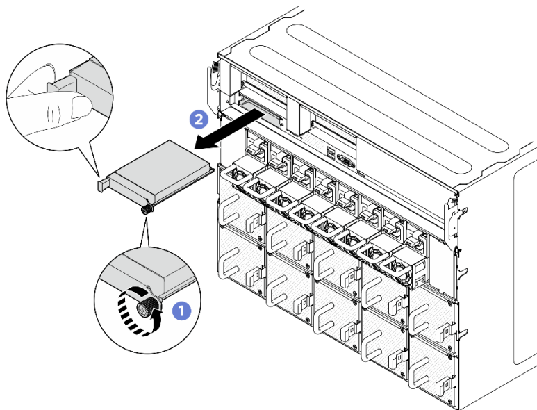
圖例 140. 卸下 OCP 模組
