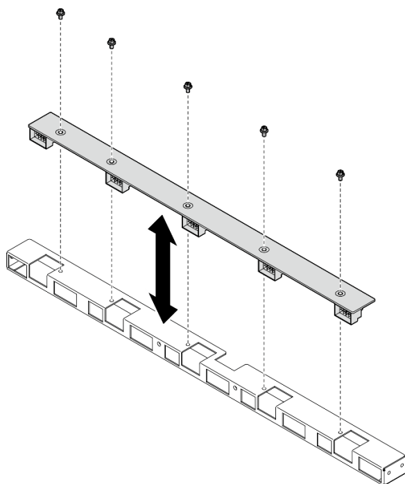
圖例 57. 卸下前方風扇控制板
