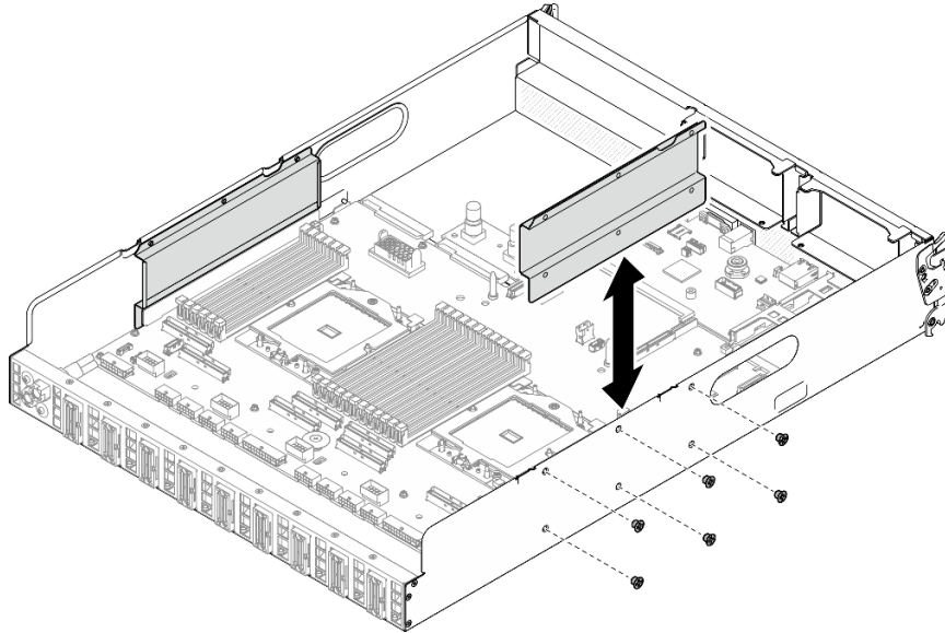
圖例 233. 安裝纜線導件
