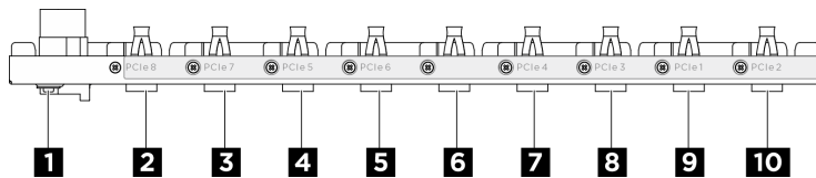
圖例 240. 後方 PCIe 交換器纜線載具纜線
