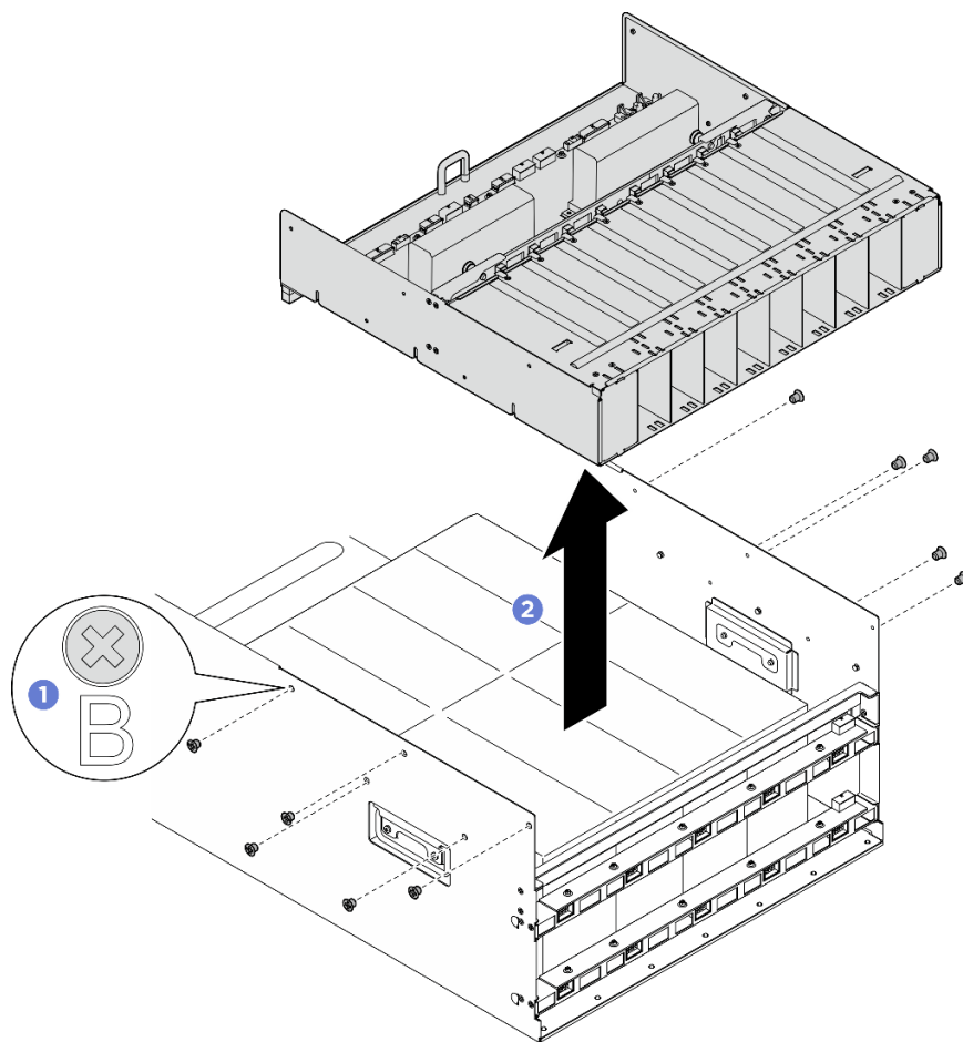
圖例 184. 卸下電源複合體
