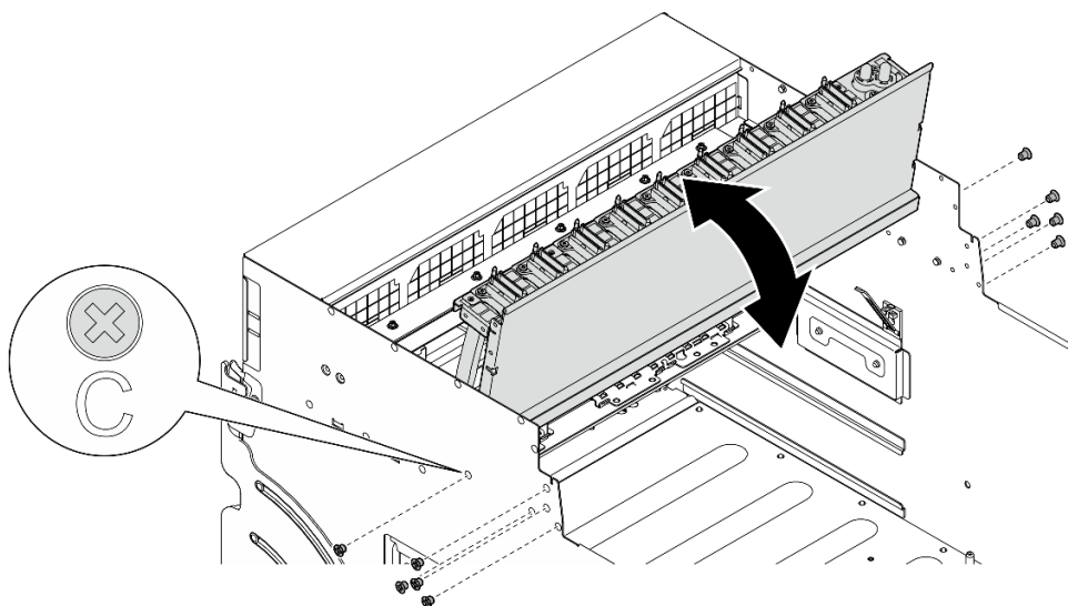
圖例 97. 翻轉前方 PCIe 交換器纜線載具
