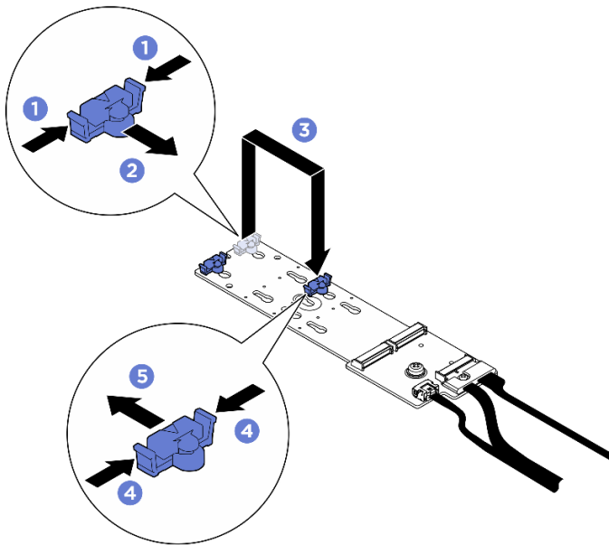
圖例 131. M.2 背板固定器調整
