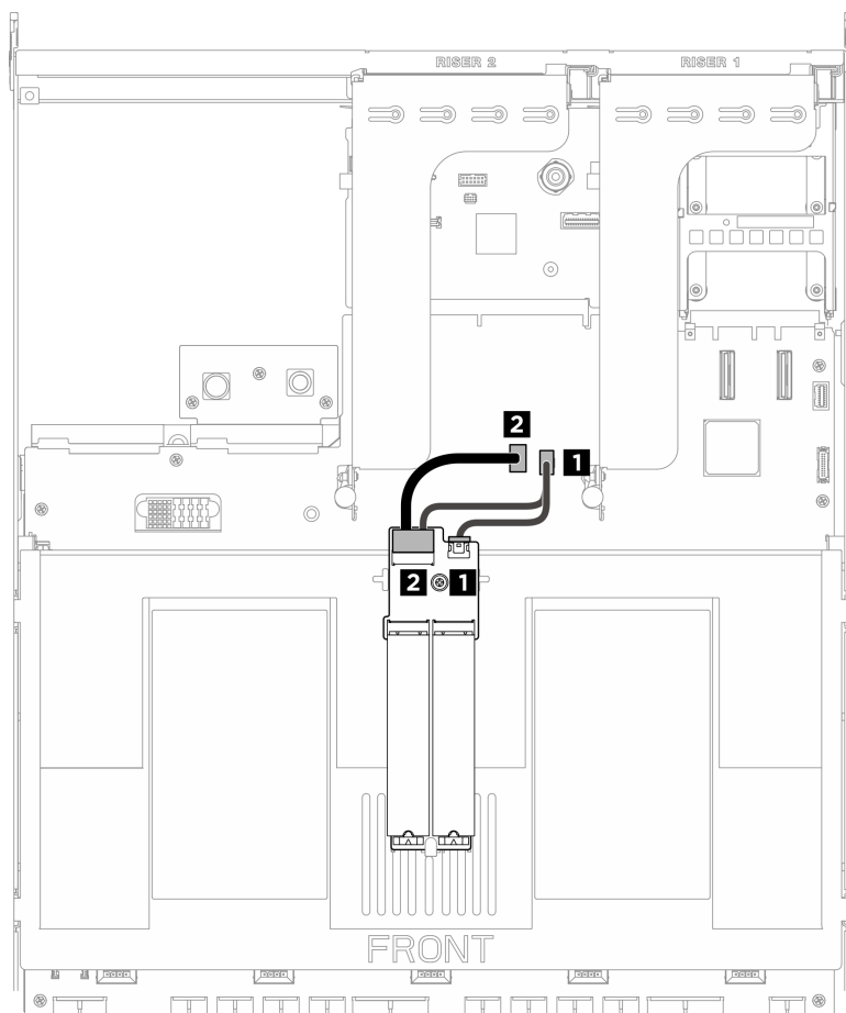
圖例 130. 連接 M.2 背板纜線
