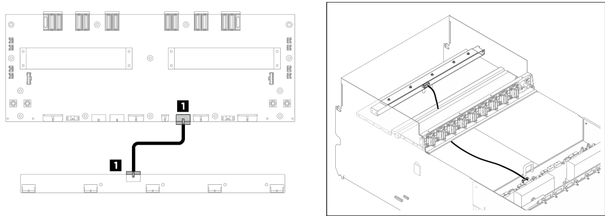
圖例 249. 前方風扇控制板纜線佈線
