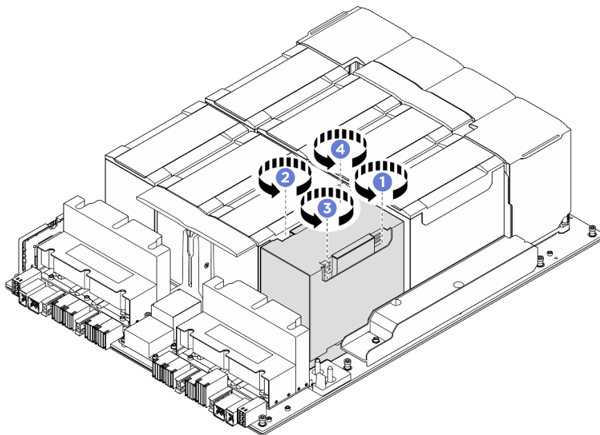
圖例 115. 螺絲鎖緊順序
