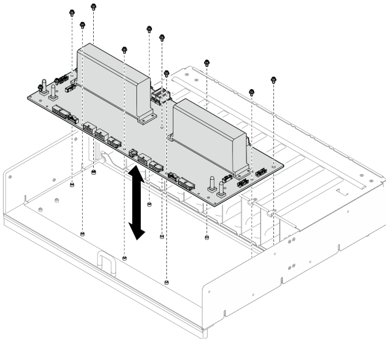
圖例 188. 安裝電源配送板
