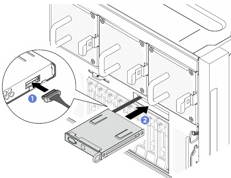
圖例 122. 安裝整合式診斷面板
