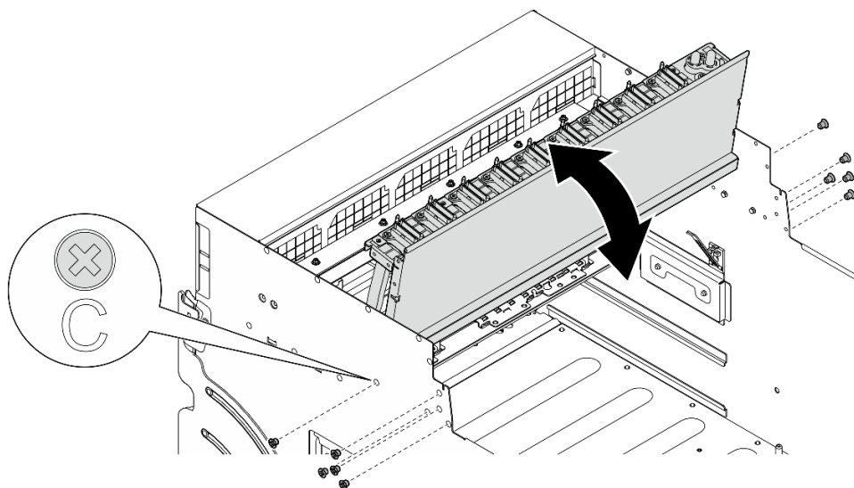
圖例 86. 翻轉前方 PCIe 交換器纜線載具
