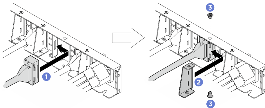
圖例 177. 安裝正面 I/O 模組、整合式診斷面板、GPU 管理或信號線
