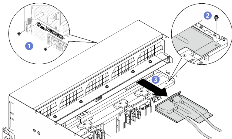
圖例 163. 卸下正面 I/O 模組
