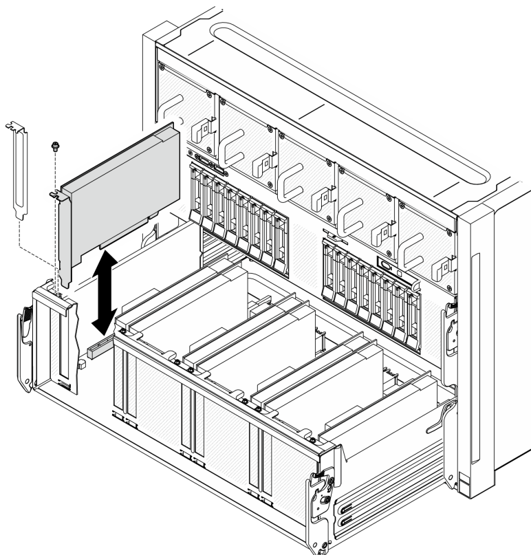
圖例 144. 安裝正面 PCIe 配接卡
