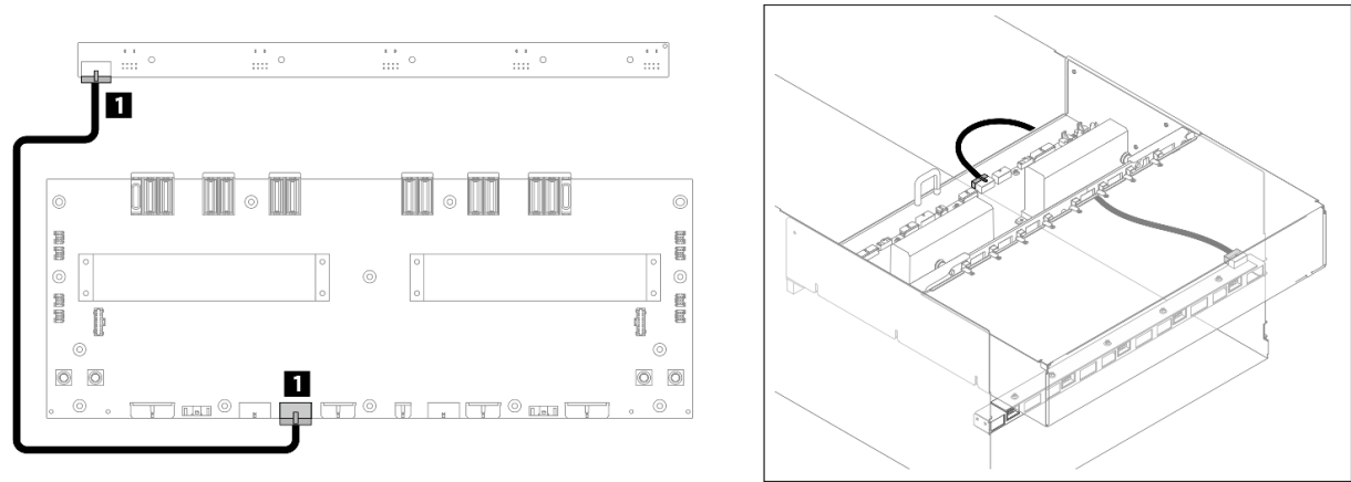
圖例 250. 後方風扇控制板（上）纜線佈線
