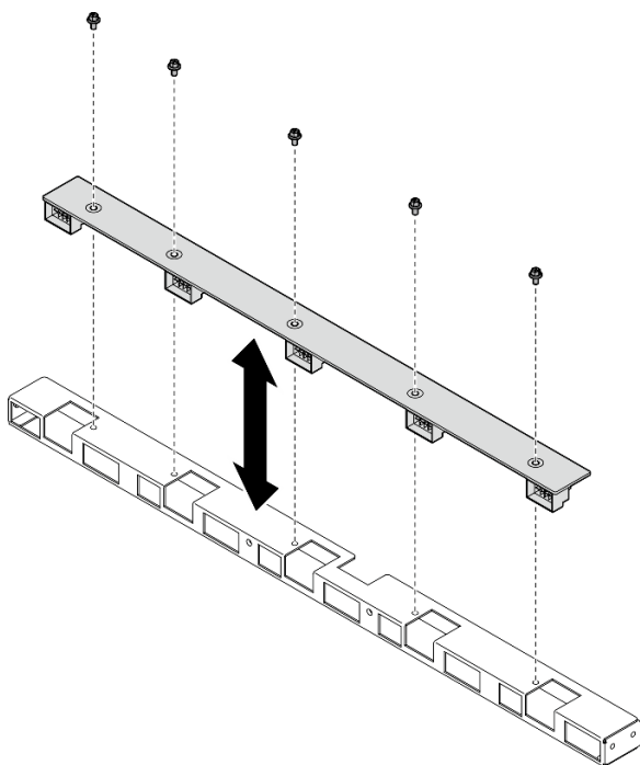
圖例 62. 卸下後方風扇控制板
