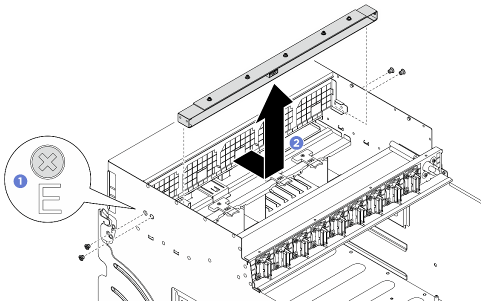
圖例 56. 卸下前方風扇控制板組件
