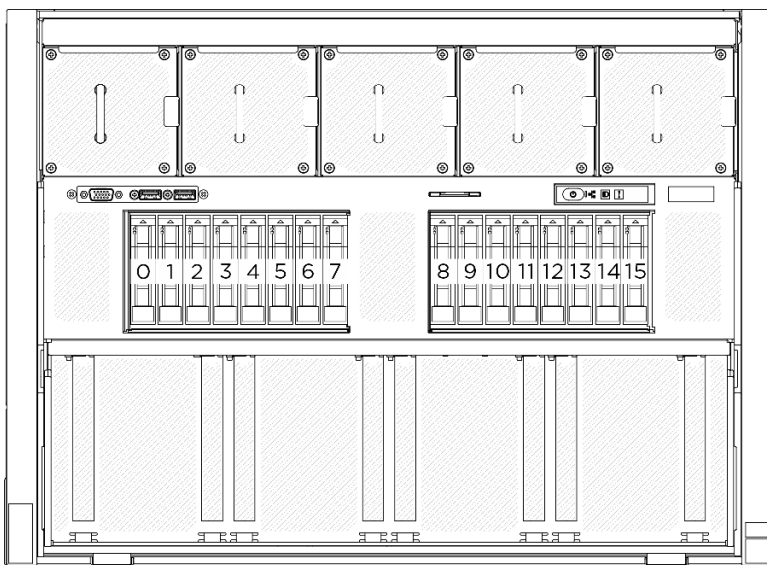
圖例 35. 2.5 吋機槽編號
