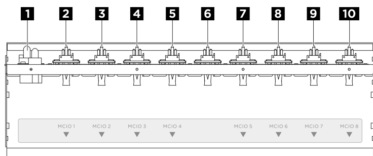
圖例 239. 前方 PCIe 交換器纜線載具纜線
