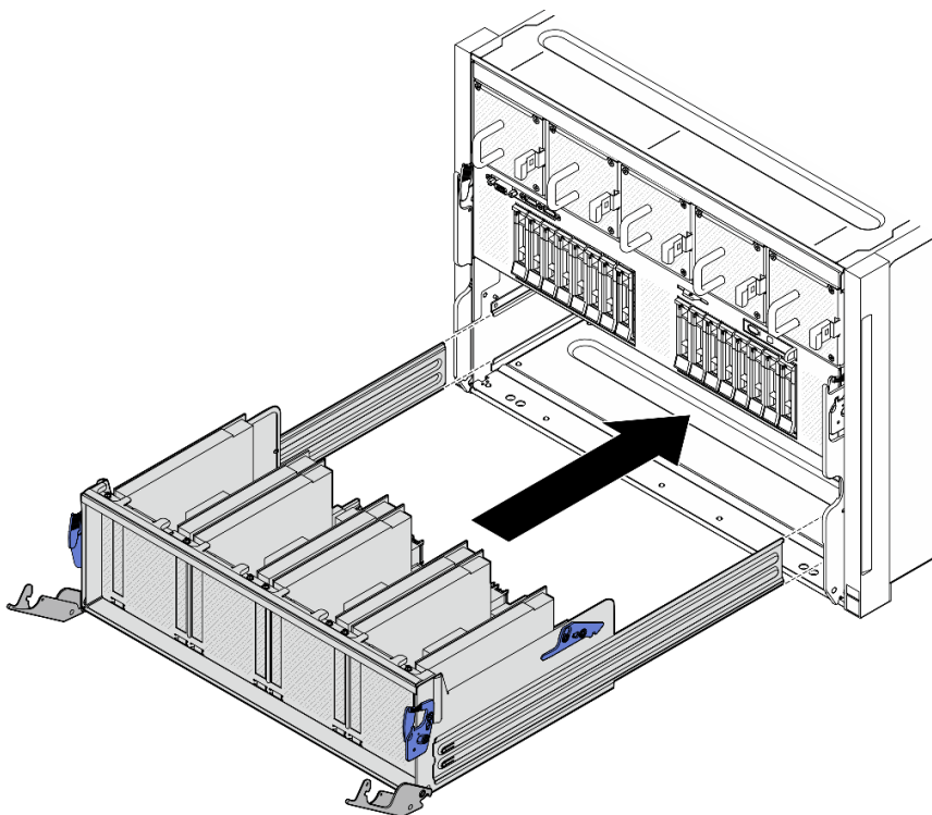
圖例 182. 將 PCIe 交換器滑動箱安裝到停止位置
