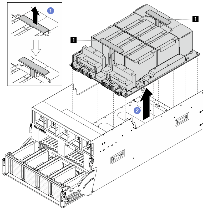
圖例 88. 卸下 GPU 複合體
