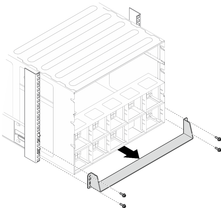
圖例 19. 卸下下支撐托架
