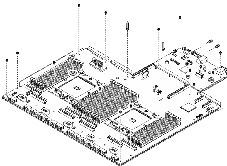
圖例 222. 卸下元件
