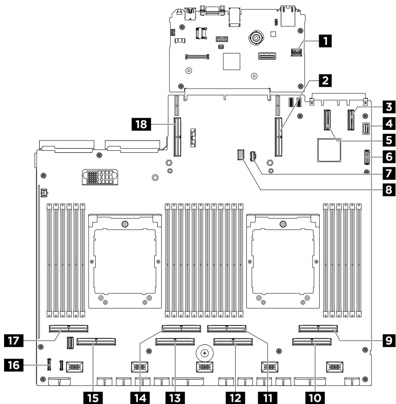
圖例 244. 用於纜線佈線的主機板組件接頭
