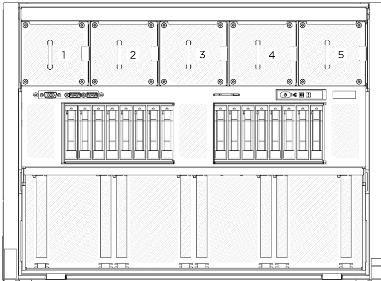
圖例 50. 前方風扇編號
