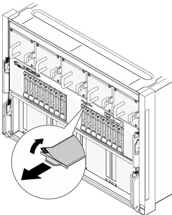
圖例 15. 拉出式資訊標籤上的 Lenovo XClarity Controller 網路存取標籤
