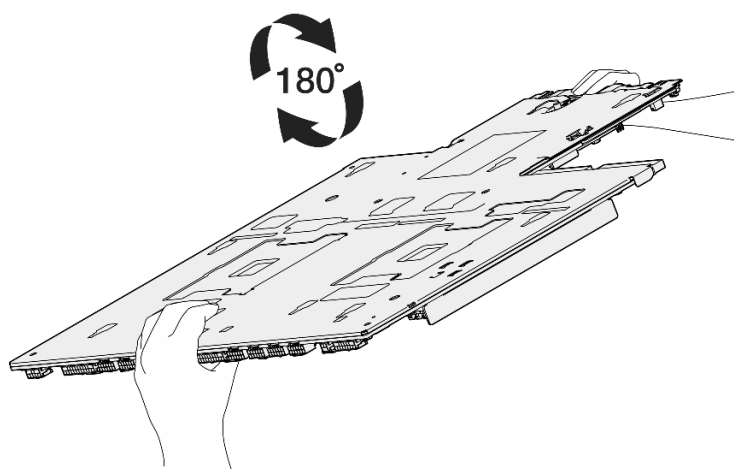
圖例 230. 將主機板組件轉至正面朝上
