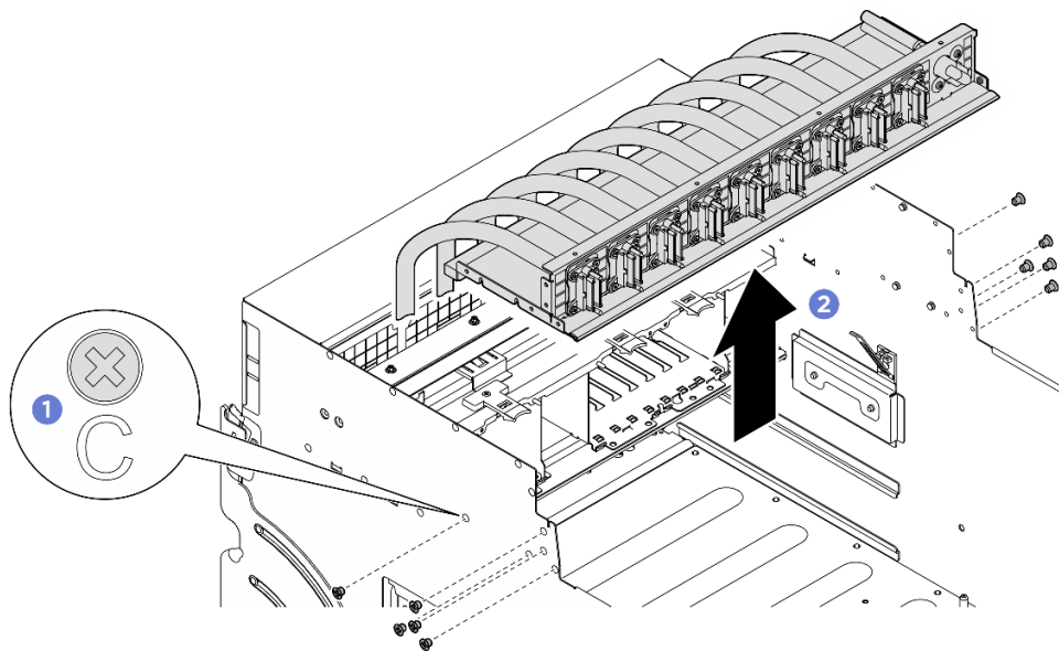
圖例 165. 卸下前方 PCIe 交換器纜線載具
