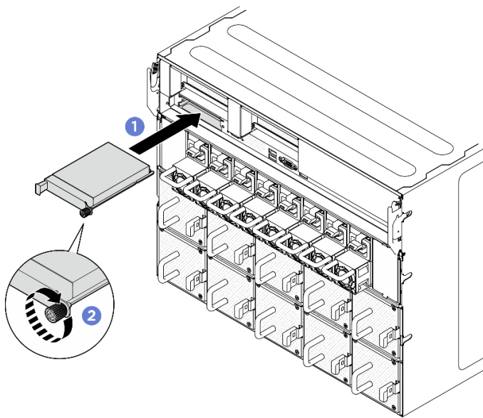
圖例 141. OCP 模組安裝
