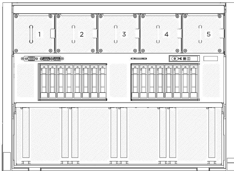
圖例 53. 前方風扇編號
