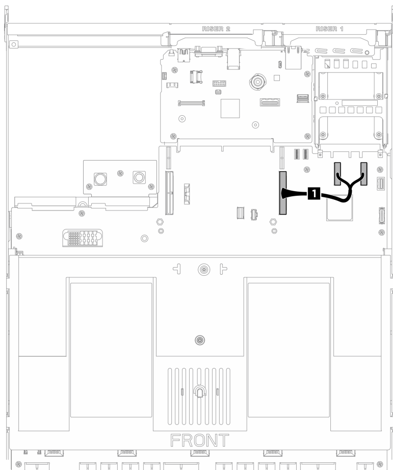
圖例 255. OCP 模組纜線佈線
