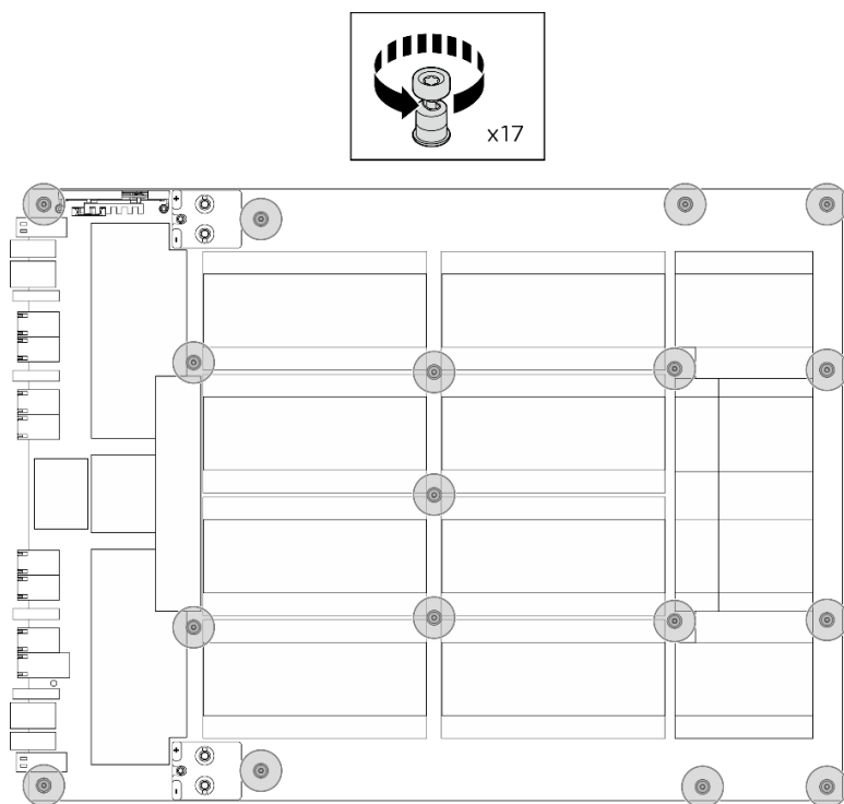
圖例 76. 卸下螺絲
