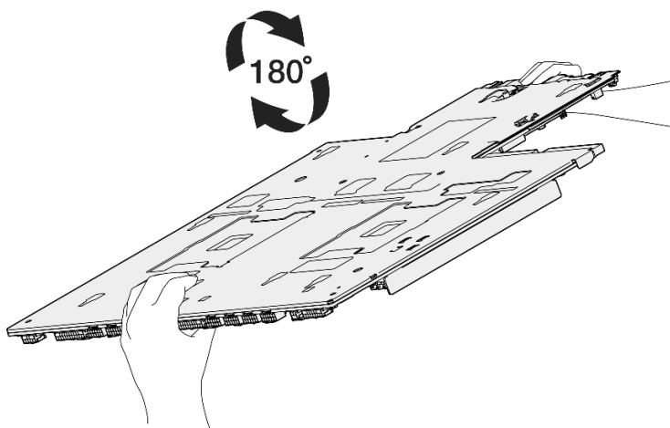
圖例 274. 將主機板組件轉至正面朝上
