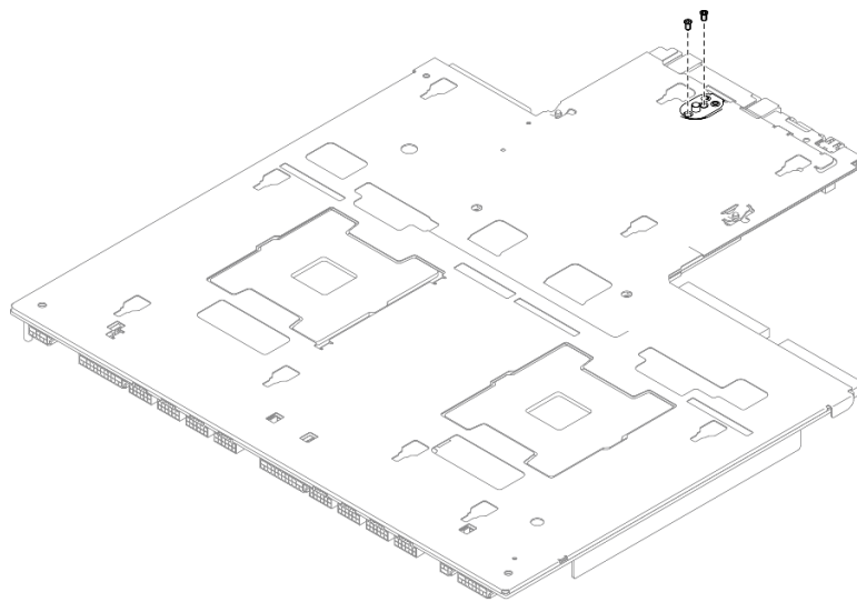
圖例 229. 安裝螺絲
