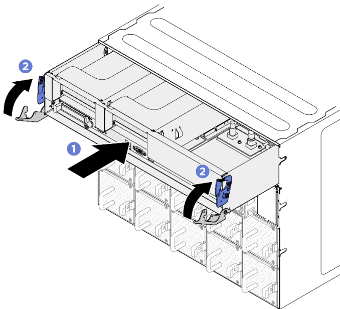
圖例 43. 安裝 2U 運算滑動箱
