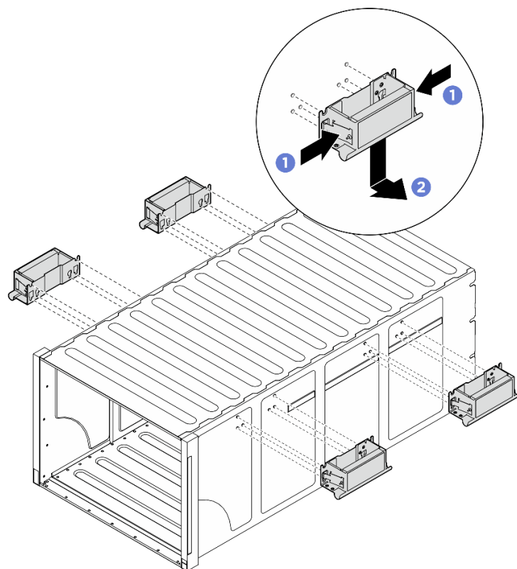
圖例 24. 卸下把手
