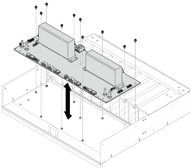
圖例 207. 卸下電源配送板
