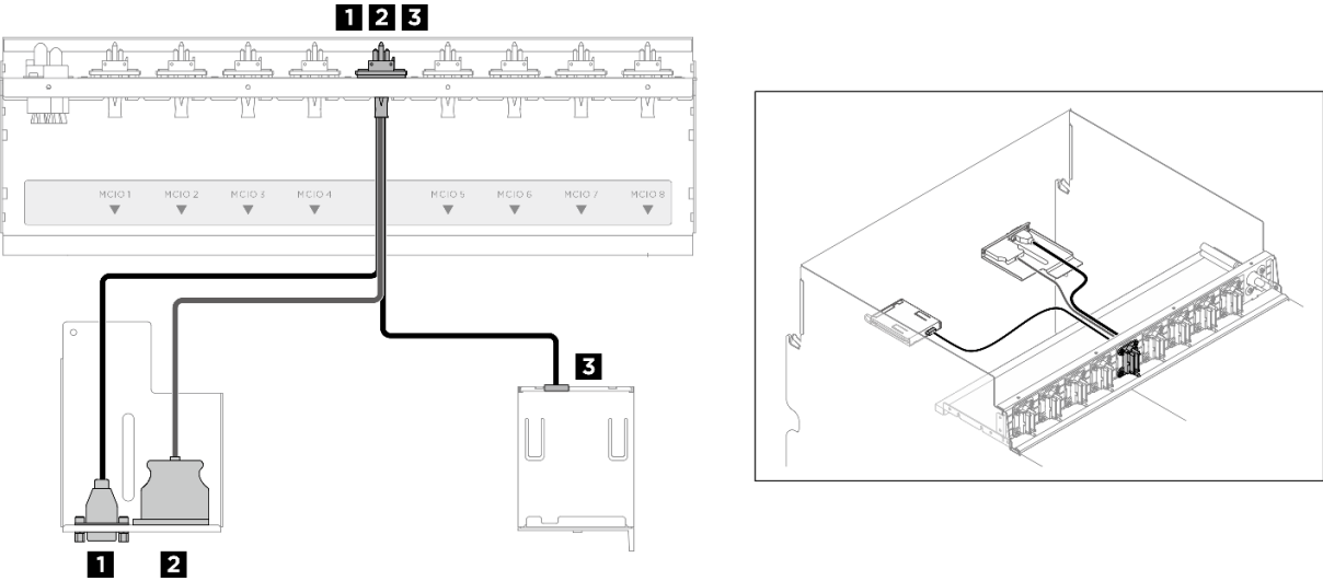
圖例 254. 正面 I/O 模組和整合式診斷面板纜線佈線
