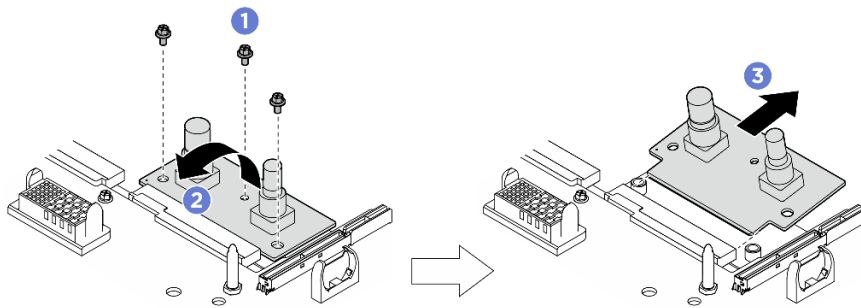
圖例 190. 電源介面板卸除
