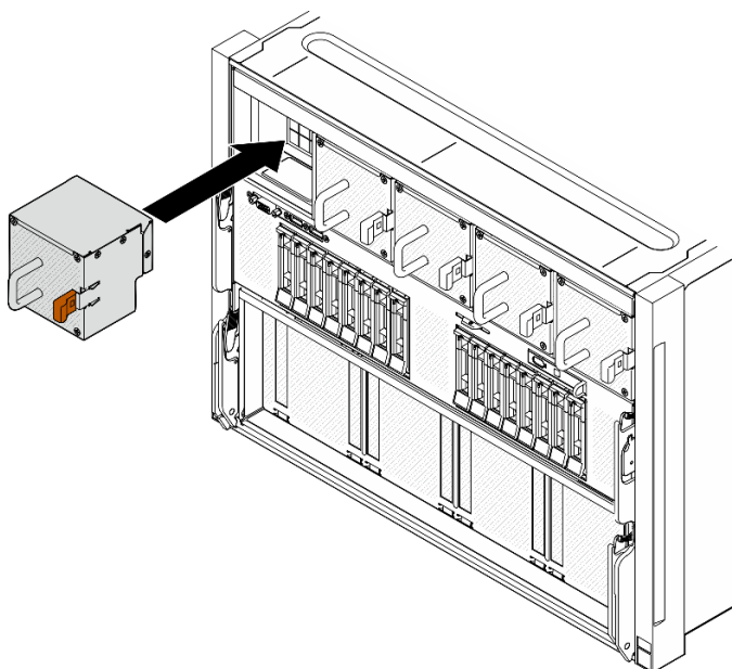
圖例 55. 安裝熱抽換風扇
