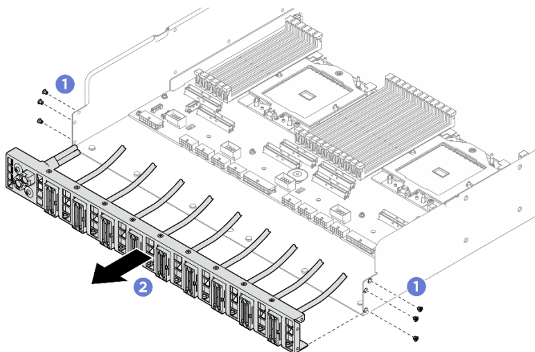
圖例 174. 卸下後方 PCIe 交換器纜線載具
