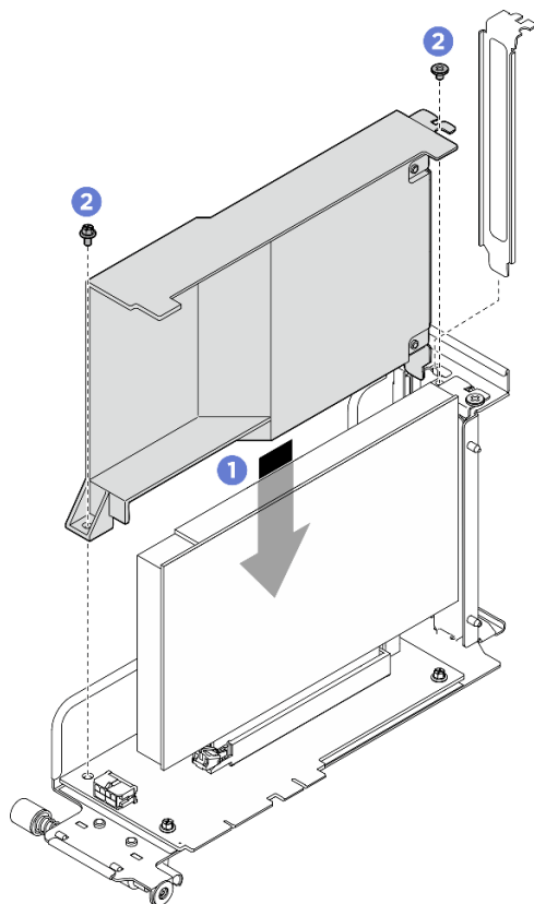
圖例 149. 安裝 PCIe 擴充卡空氣擋板
