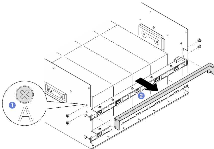
圖例 95. 卸下後支撐托架
