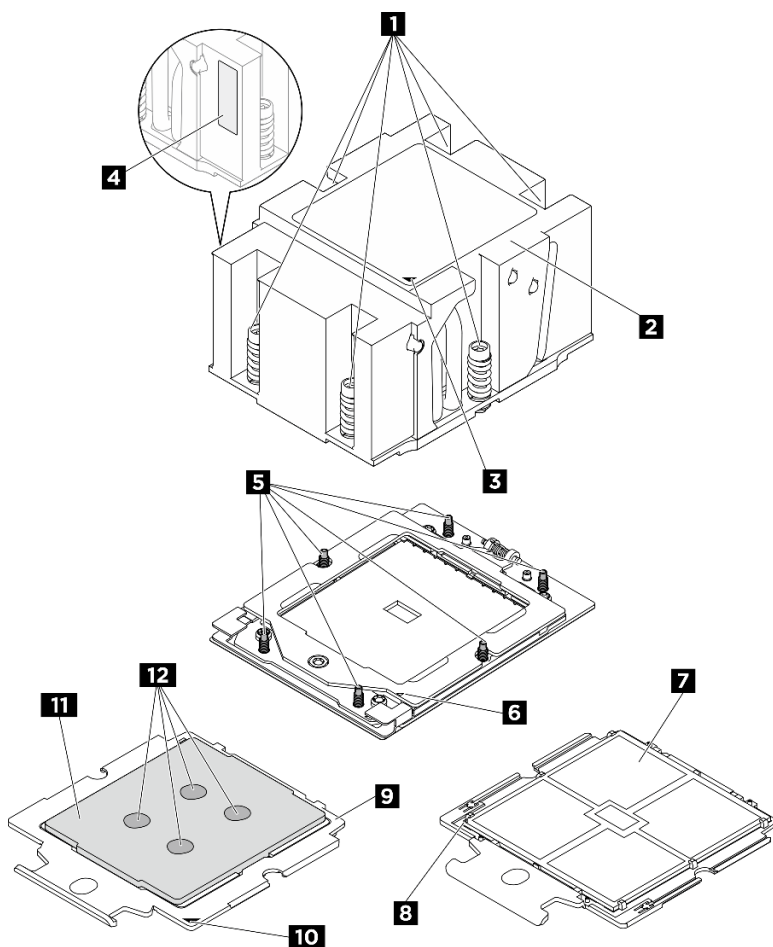
圖例 199. 處理器和散熱槽元件
