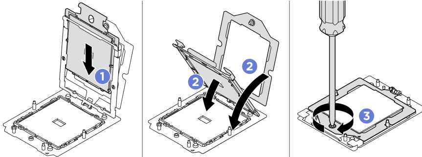
圖例 202. 安裝處理器
