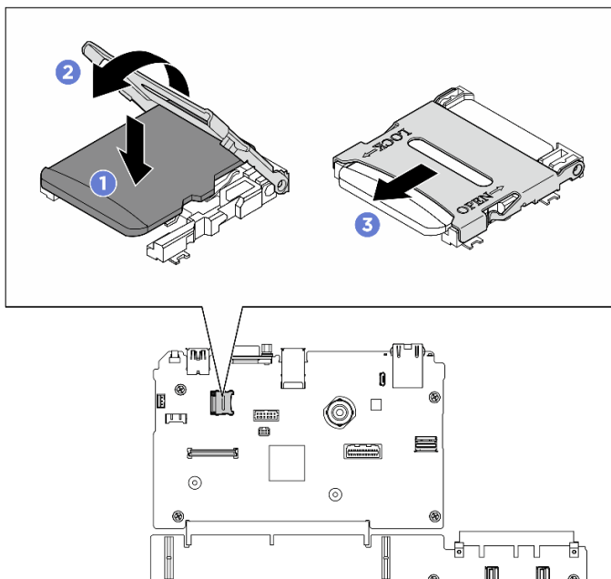
圖例 139. 安裝 MicroSD 卡
