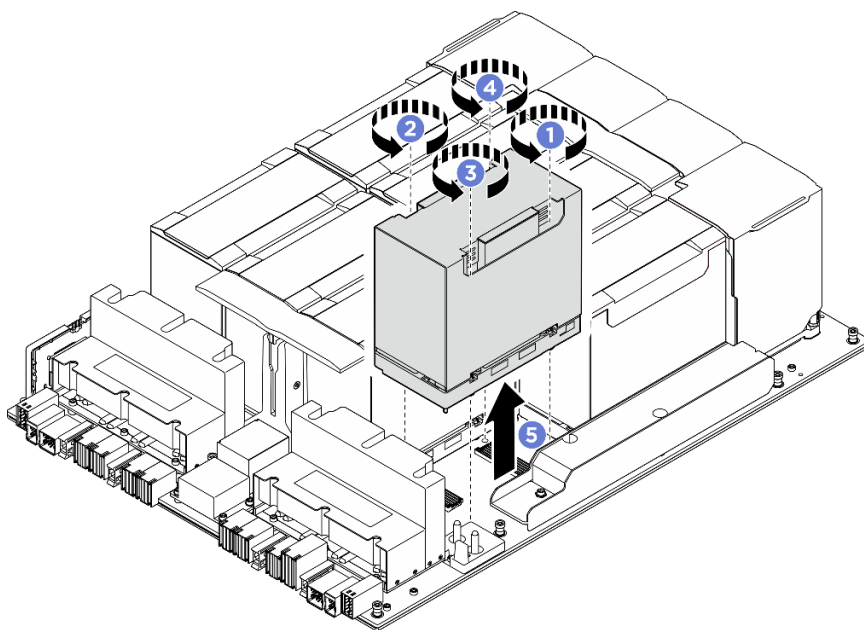
圖例 113. 卸下 GPU 和散熱槽模組
