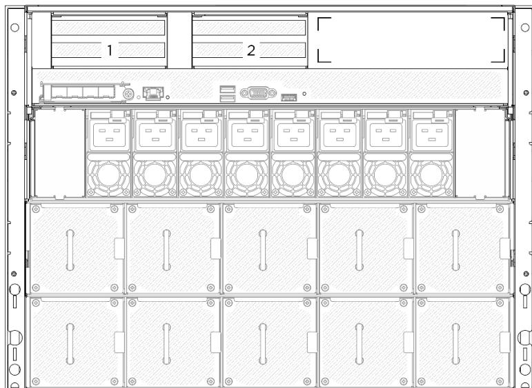
圖例 150. PCIe 擴充卡位置
