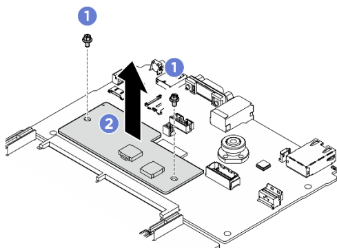
圖例 214. 卸下韌體和 RoT 安全模組
