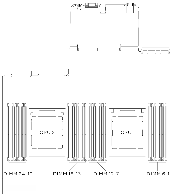
圖例 134. 記憶體模組和處理器佈置
