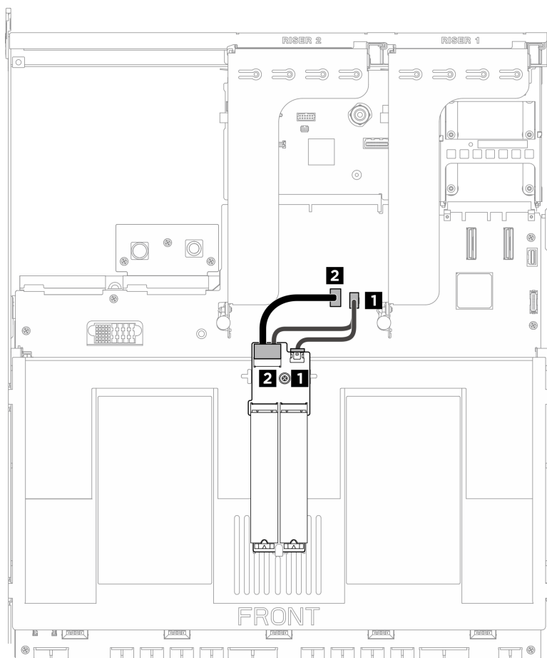
圖例 198. 連接 M.2 背板纜線
