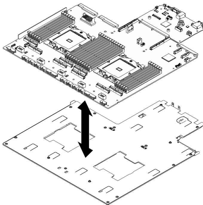
圖例 223. 拆卸主機板組件
