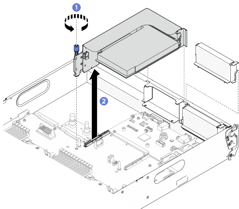
圖例 151. 卸下 PCIe 擴充卡組件
