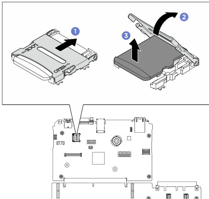
圖例 138. 卸下 MicroSD 卡
