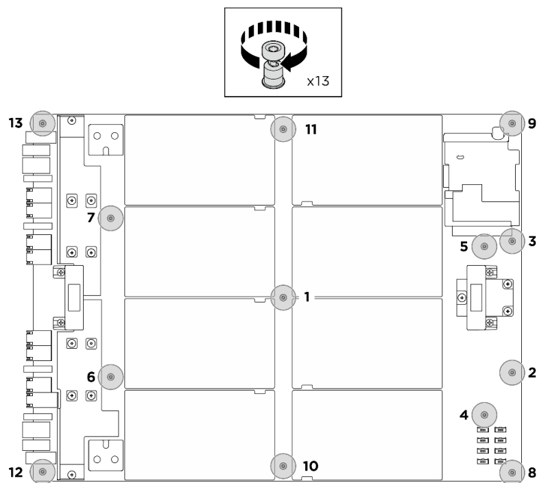
圖例 101. 安裝螺絲
