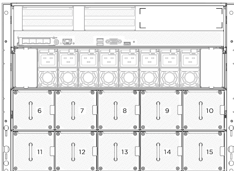
圖例 51. 後方風扇編號
