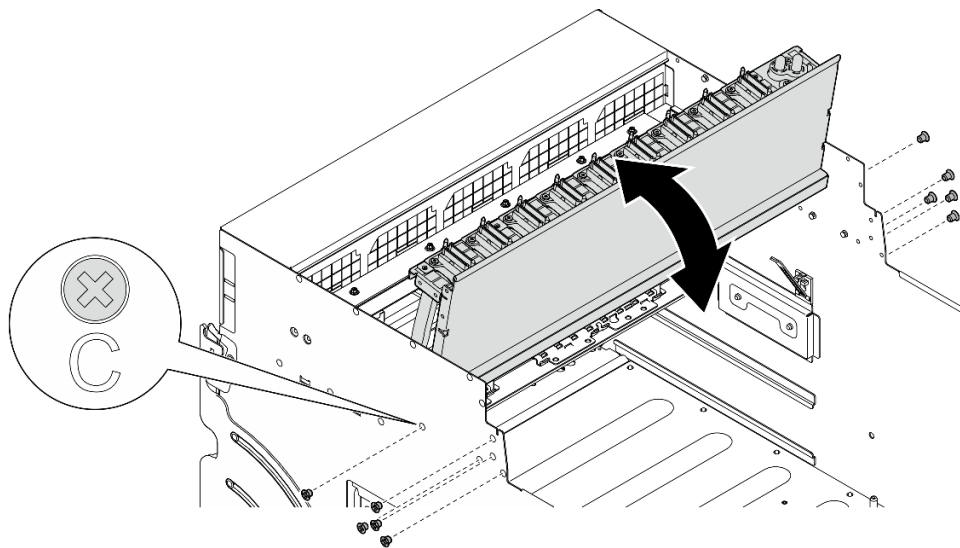
圖例 75. 翻轉前方 PCIe 交換器纜線載具
