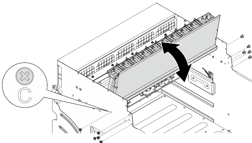
圖例 109. 翻轉前方 PCIe 交換器纜線載具
