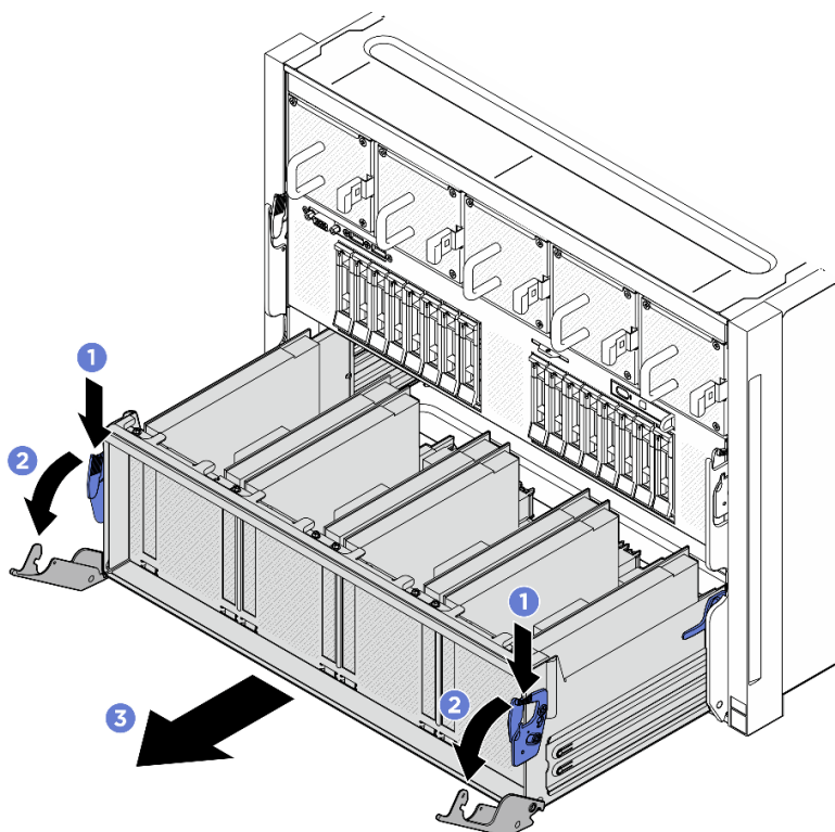
圖例 105. 將 PCIe 交換器滑動箱拉動到停止位置
