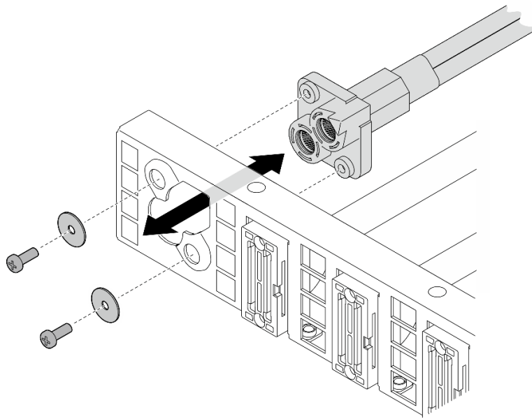
圖例 176. 卸下電源線
