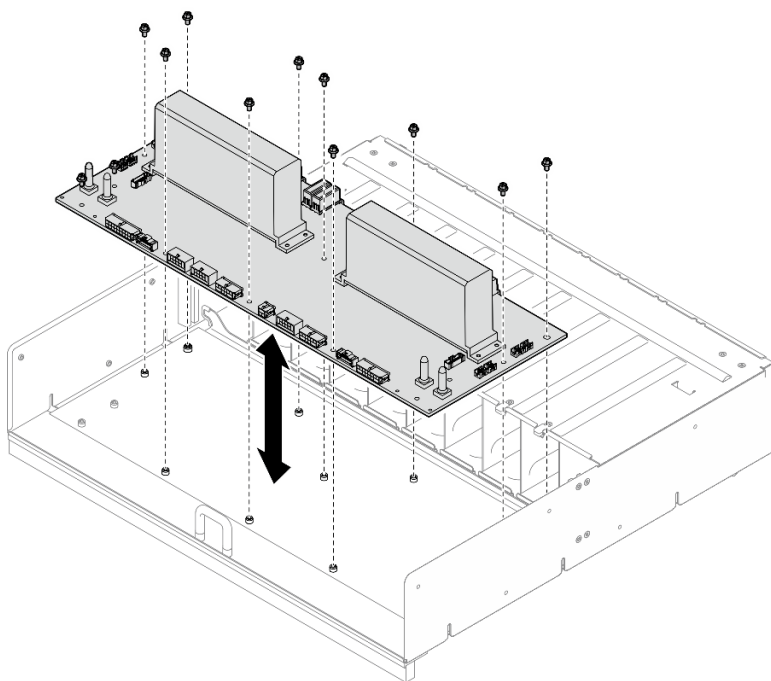
圖例 187. 卸下電源配送板
