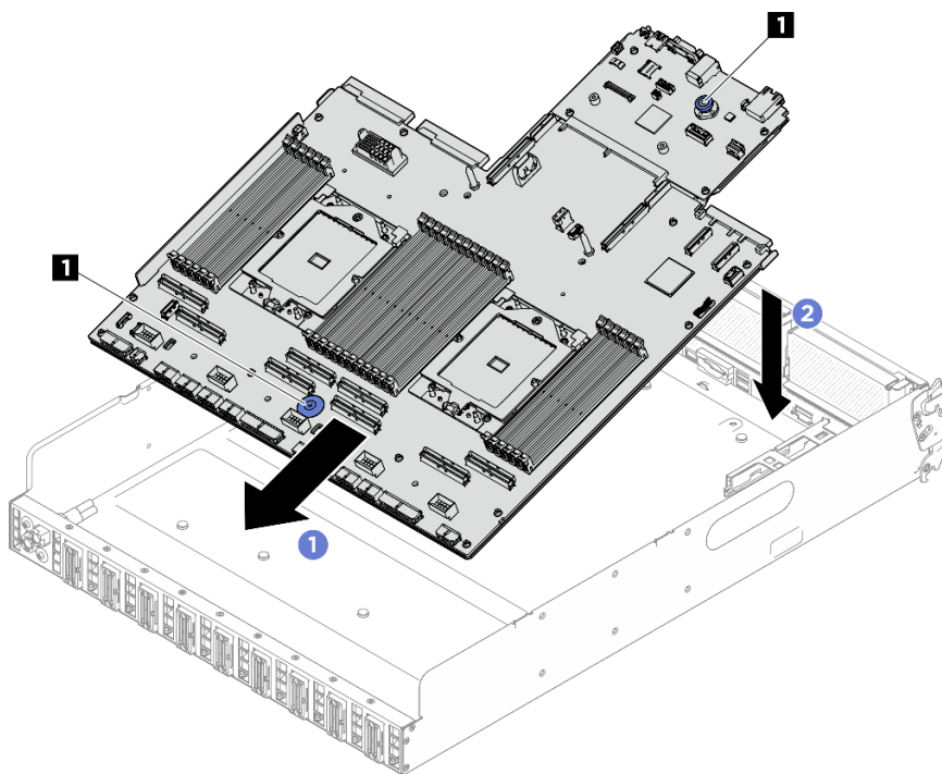
圖例 231. 安裝主機板組件
