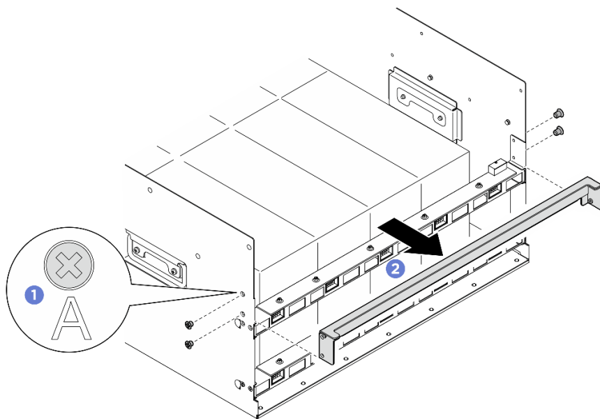
圖例 104. 卸下後支撐托架
