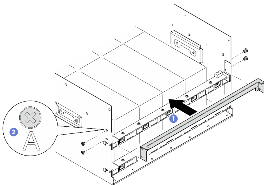
圖例 103. 安裝後支撐托架
