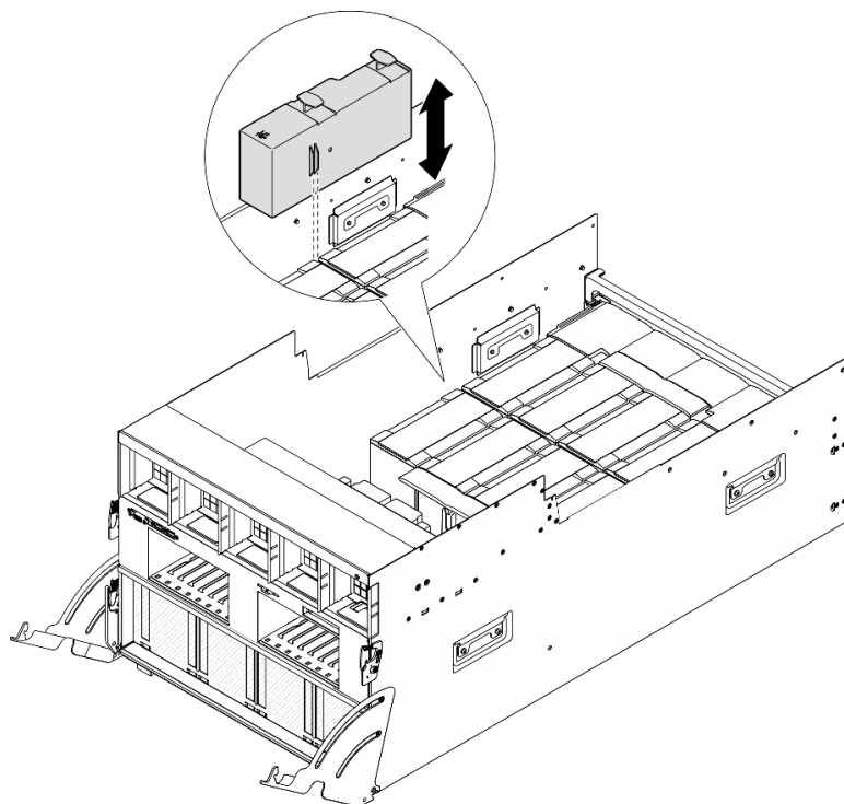
圖例 69. 卸下 GPU 空氣導管
