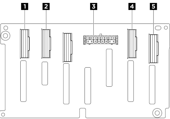
圖例 234. 2.5 吋 NVMe 背板接頭
