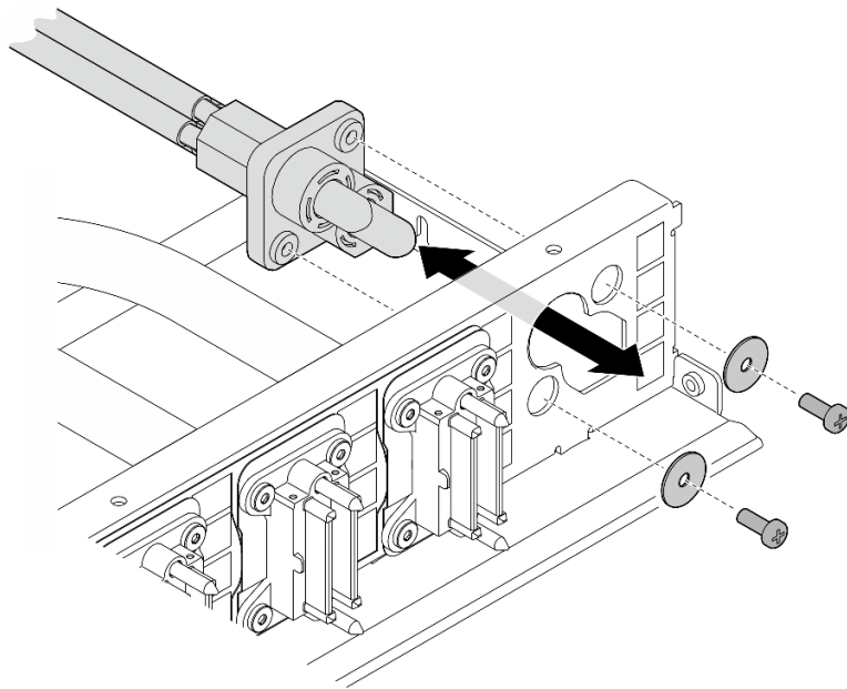
圖例 167. 卸下電源線
