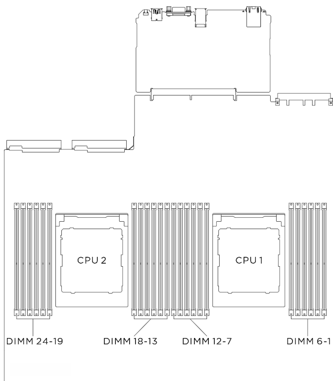
圖例 136. 記憶體模組和處理器佈置
