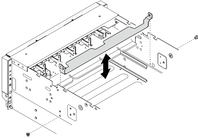
圖例 95. 卸下 GPU 接頭保護托架
