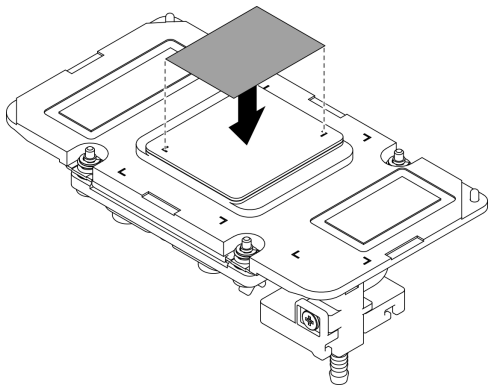
圖例 231. 貼附 PCM
