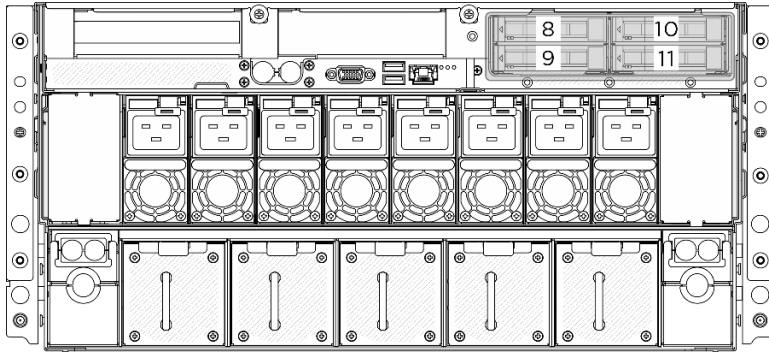
圖例 352. 後方 2.5 吋硬碟背板編號
