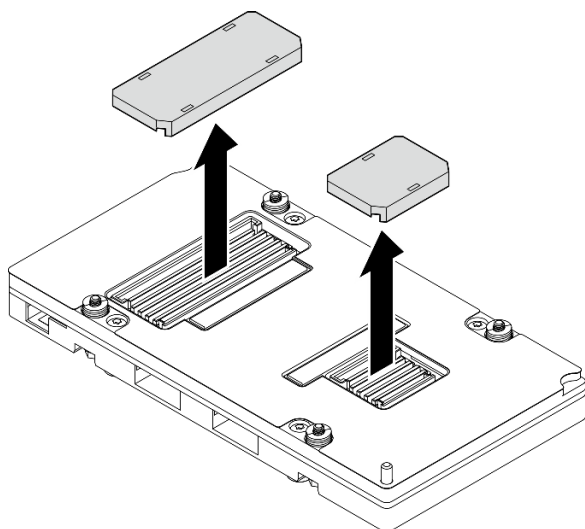
圖例 205. 移除接頭蓋
