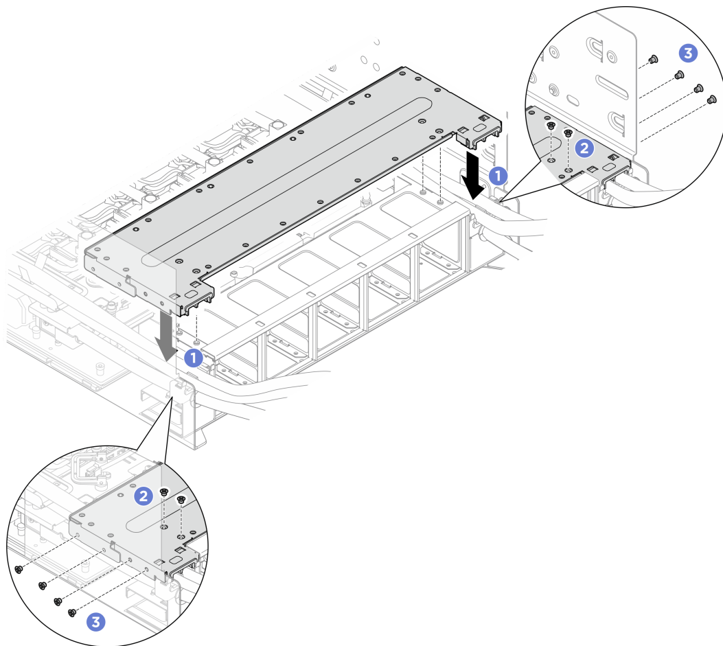
圖例 134. 安裝後方風扇機盒支撐托架
