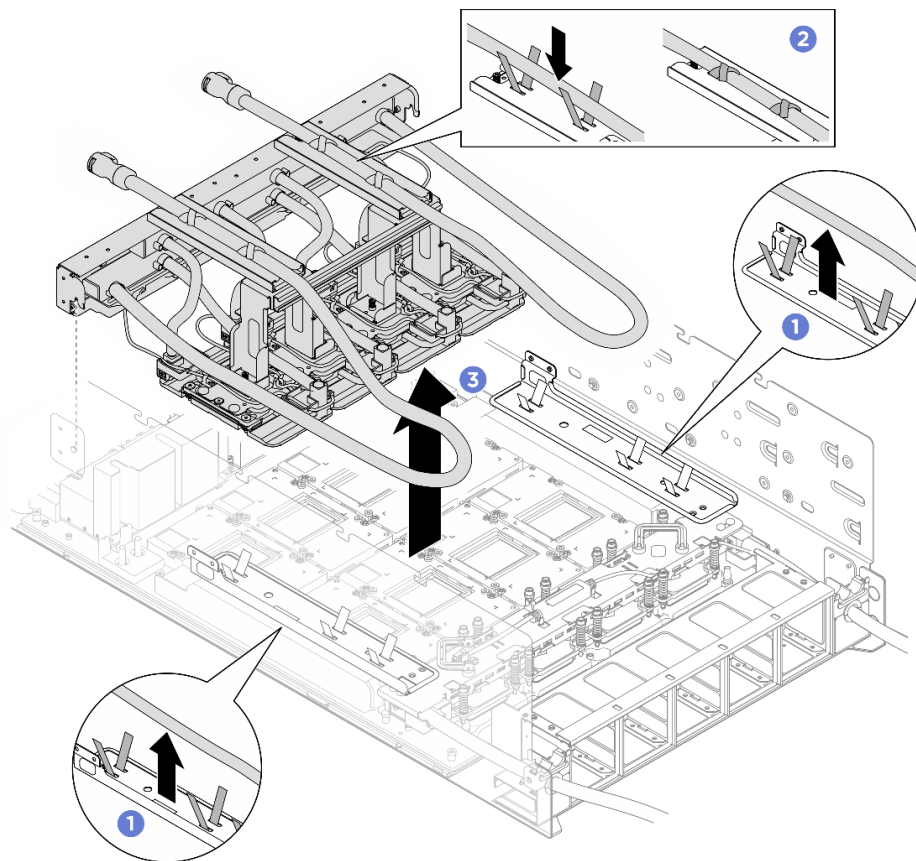
圖例 144. 卸下前方 H100/H200 GPU 水冷板模組
