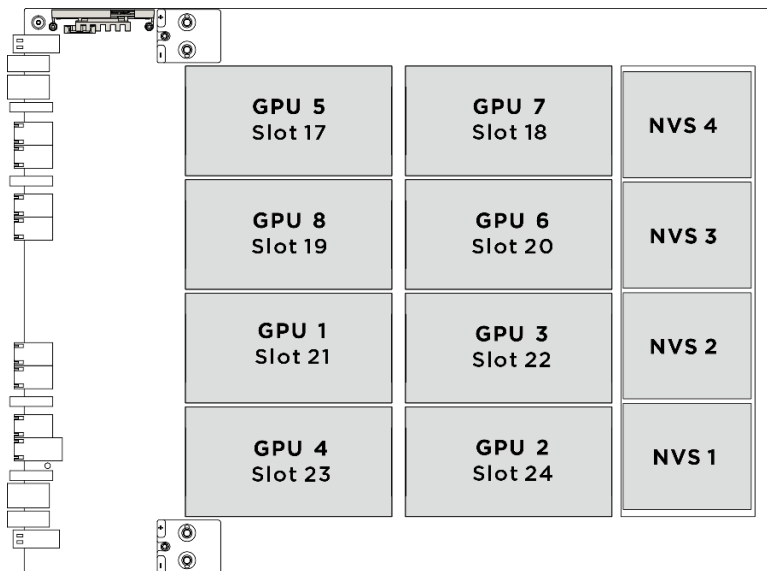
圖例 112. GPU 編號
