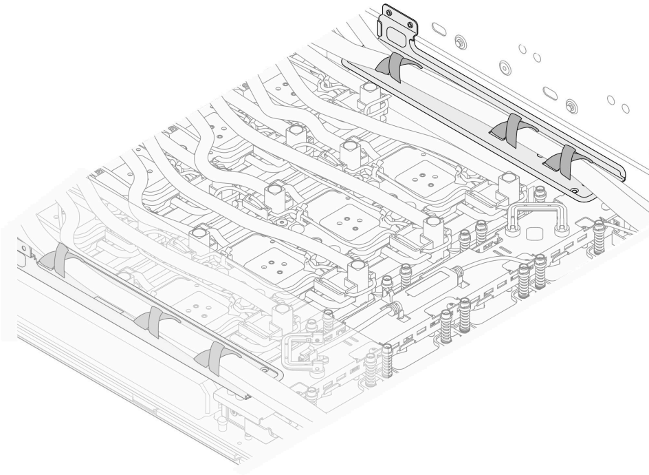
圖例 186. 用軟管束帶固定軟管和纜線
