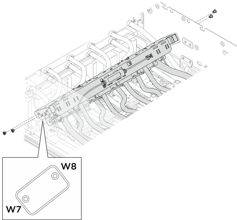
圖例 139. 卸下後方 H100/H200 GPU 水冷板模組歧管
