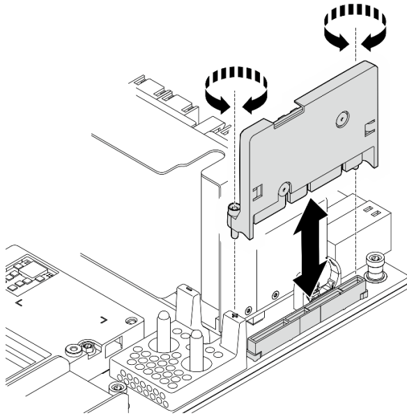
圖例 239. 卸下 HMC 卡
