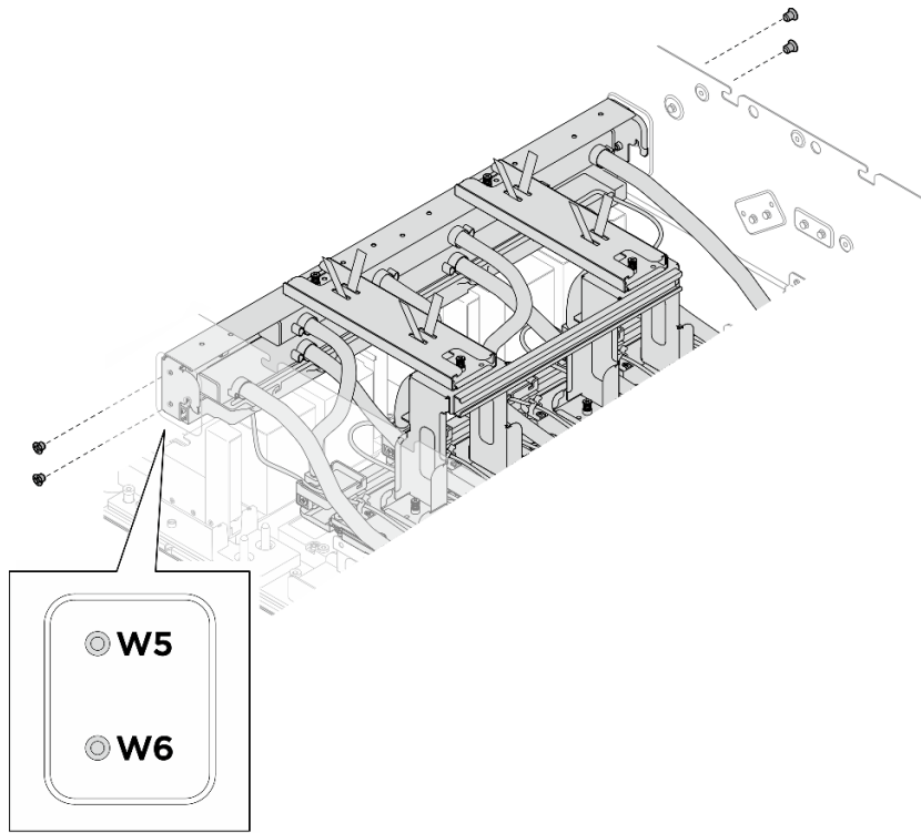
圖例 143. 卸下前方 H100/H200 GPU 水冷板模組歧管
