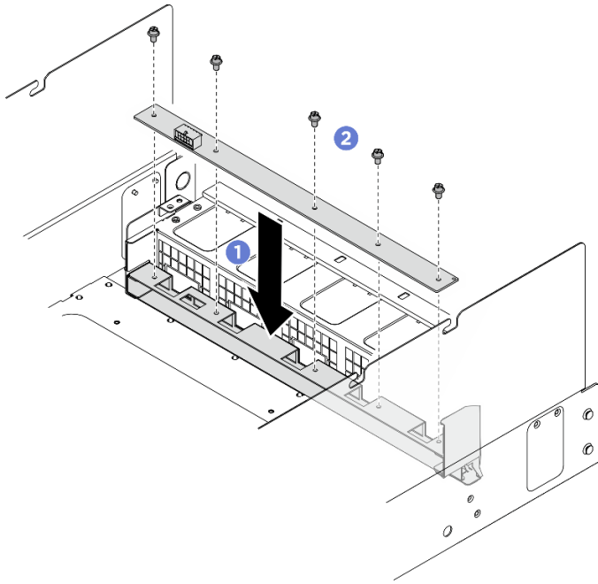
圖例 68. 安裝後方風扇控制板
