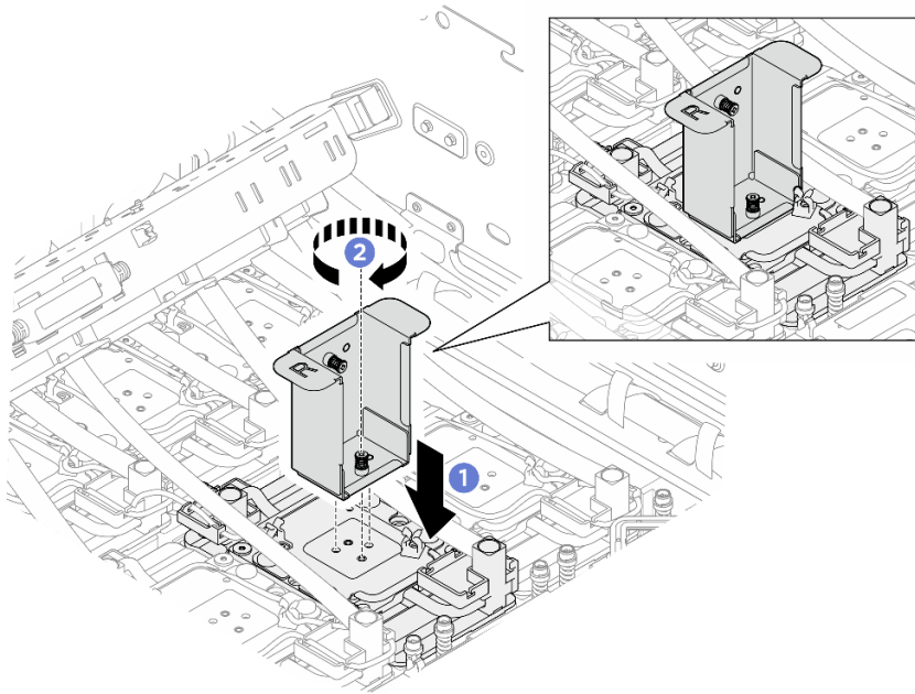
圖例 222. 將維修托架安裝到 GPU 水冷板上
