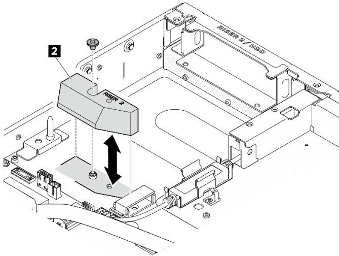
圖例 35. 從機箱卸下 DPU 空氣擋板
