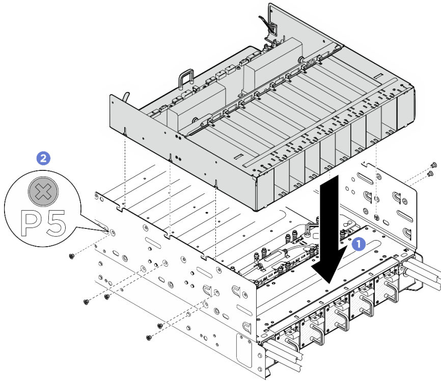
圖例 321. 安裝電源複合體
