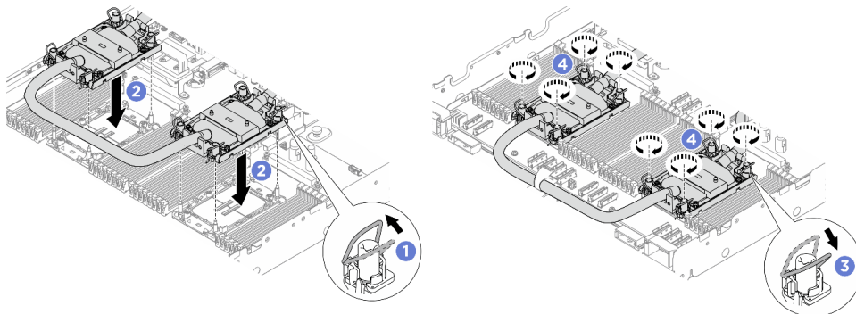
圖例 265. 安裝處理器連接 DWCM
