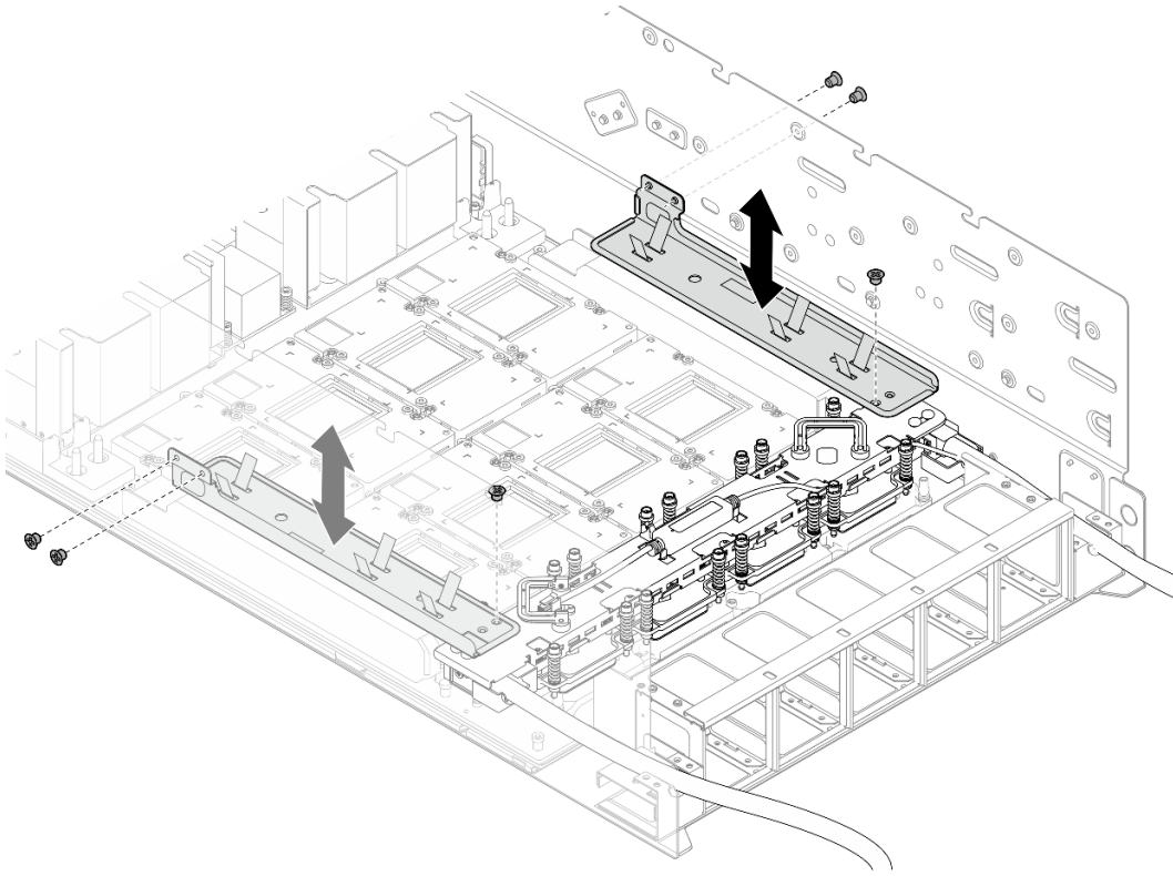
圖例 132. 安裝軟管導管
