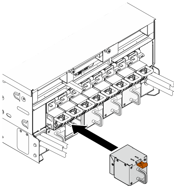
圖例 59. 後方風扇安裝
