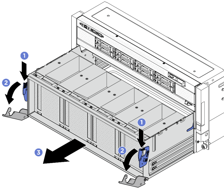
圖例 313. 將 PCIe 交換器滑動箱從停止位置卸下
