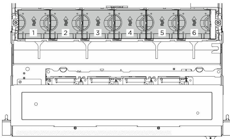
圖例 49. 前方風扇編號
