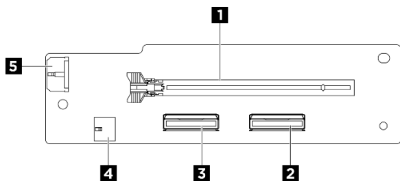
圖例 374. PCIe 擴充卡接頭
