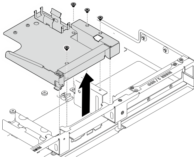
圖例 246. 卸下洩漏感應器模組托架
