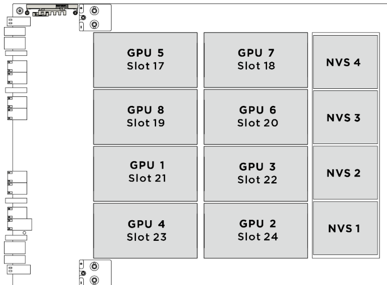
圖例 219. GPU 編號
