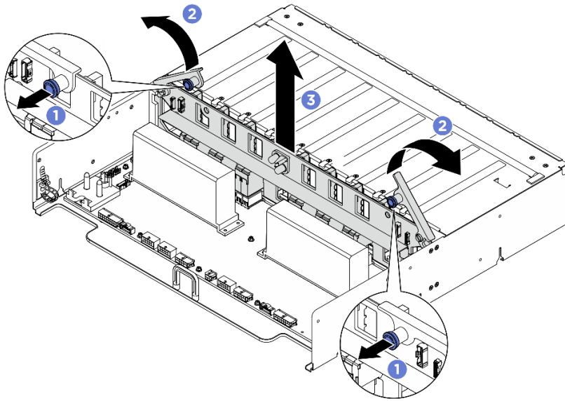
圖例 323. 卸下 PSU 轉插卡
