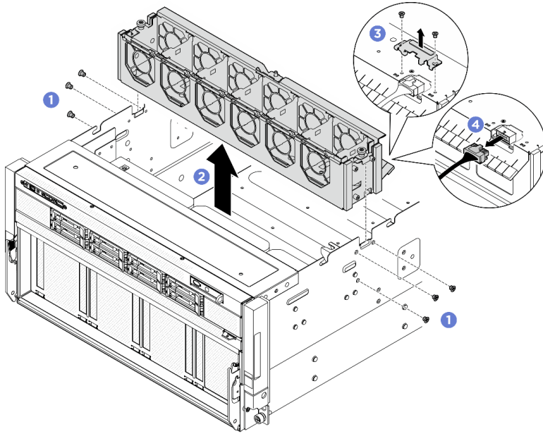
圖例 51. 卸下風扇機盒
