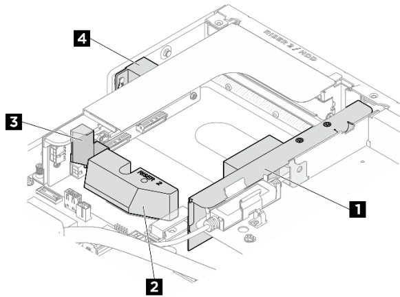
圖例 43. DPU 空氣擋板在擴充卡 2 插槽中的位置
