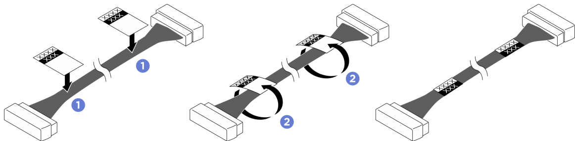
圖例 329. 黏貼標籤
