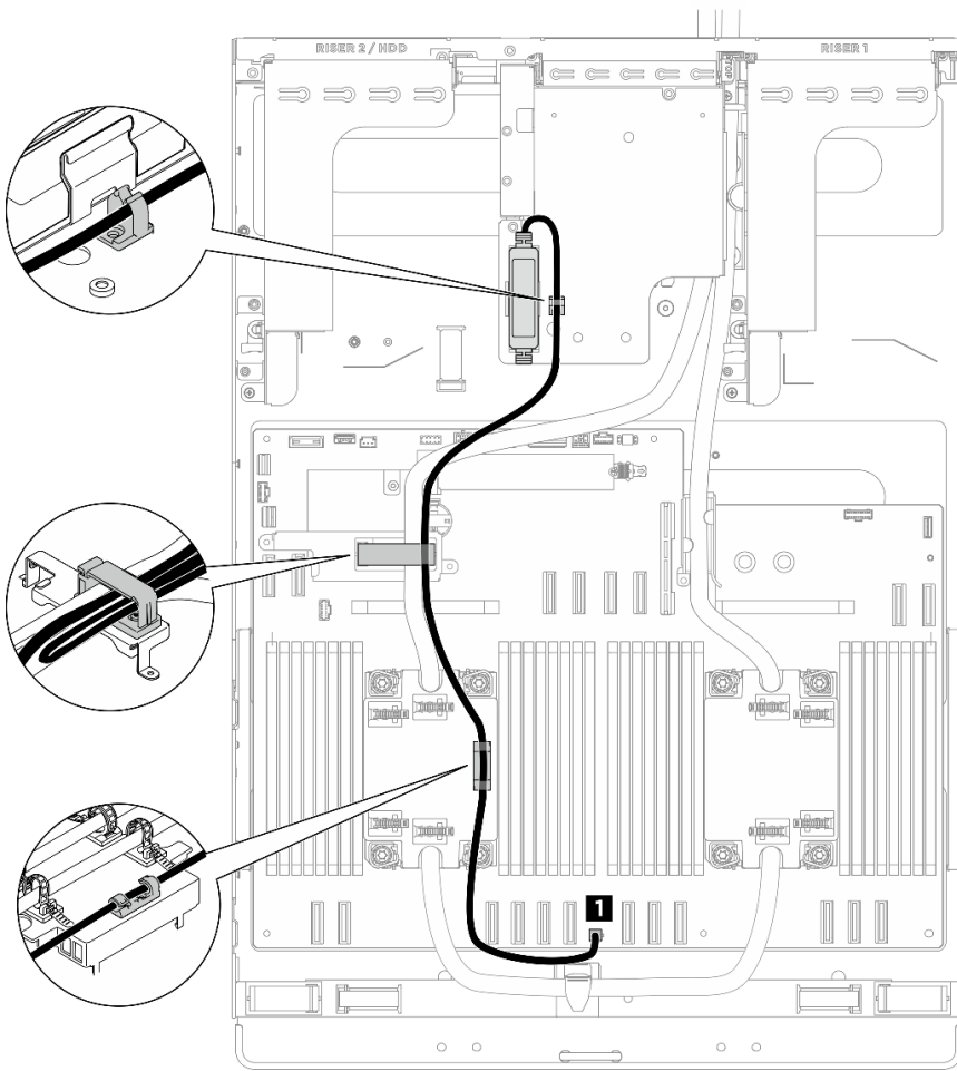
圖例 400. DWCM 洩漏感應器模組纜線佈線
