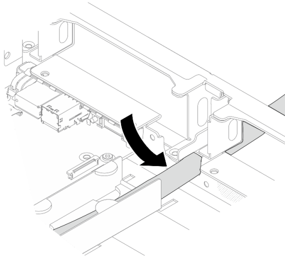
圖例 269. 安裝軟管
