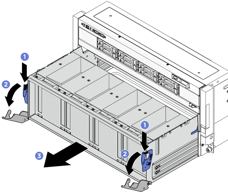
圖例 77. 將 PCIe 交換器滑動箱從停止位置卸下
