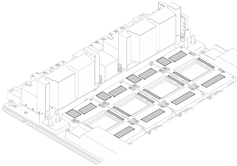
圖例 145. 清除 GPU 上的 PCM 和油灰墊
