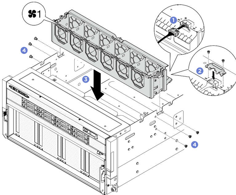
圖例 52. 安裝風扇機盒
