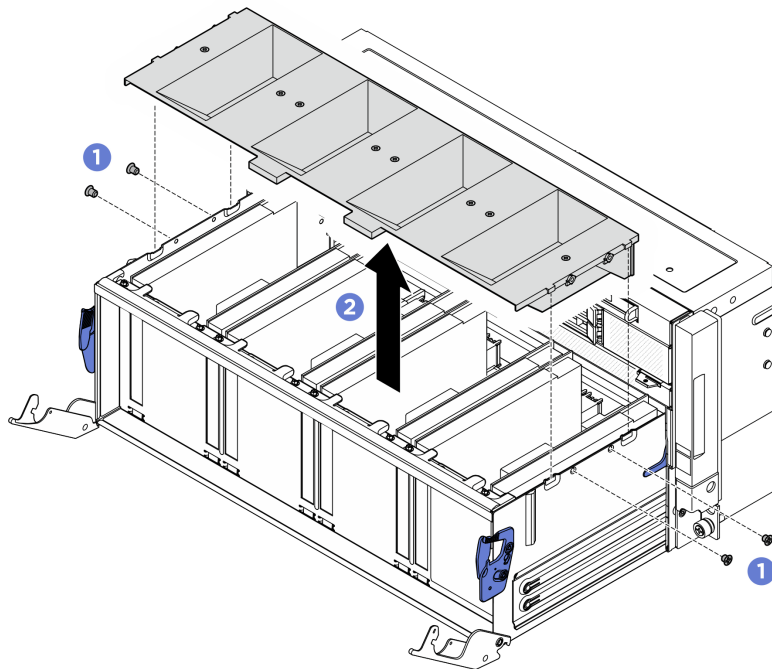
圖例 314. 卸下空氣擋板
