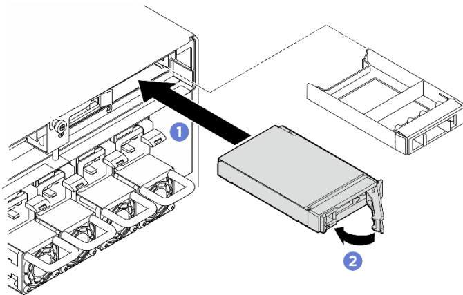
圖例 15. 安裝背面 2.5 吋熱抽換硬碟
