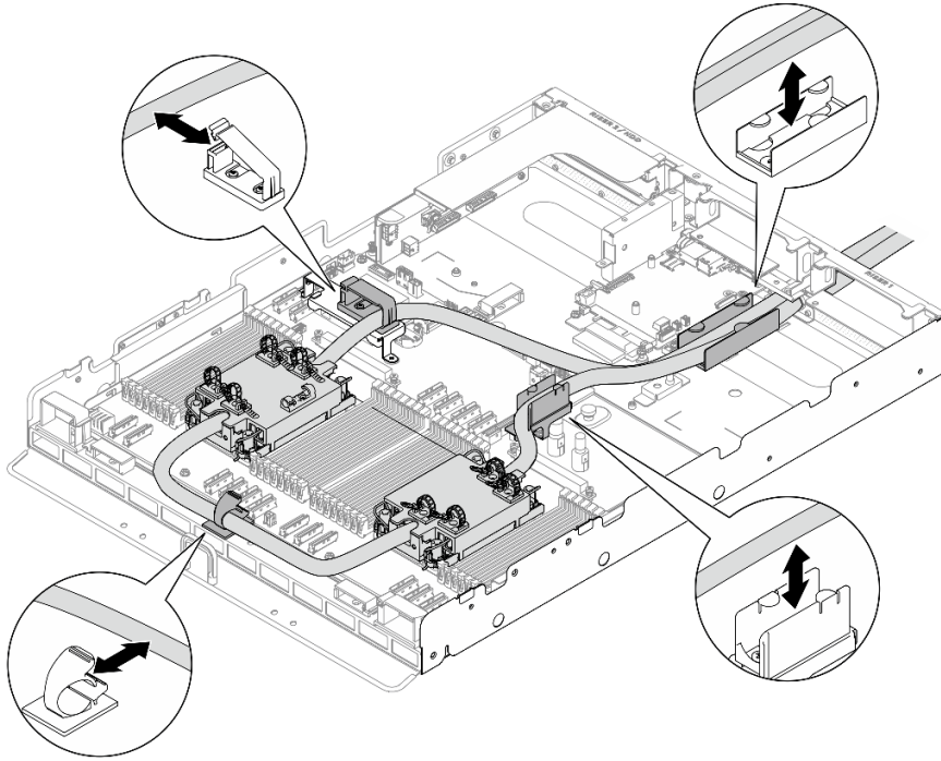
圖例 268. 安裝軟管和模組
