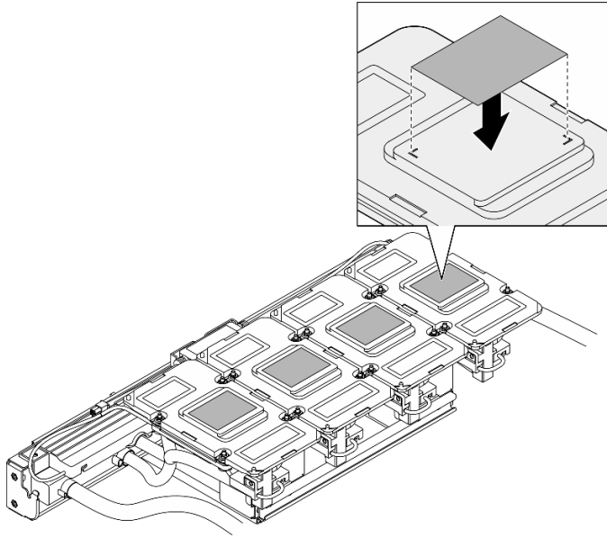
圖例 151. 貼附 PCM
