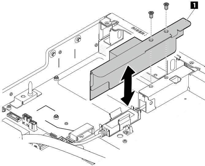
圖例 45. 安裝 DPU 空氣擋板和托架組件
