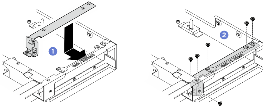
圖例 356. 安裝背面框架托架
