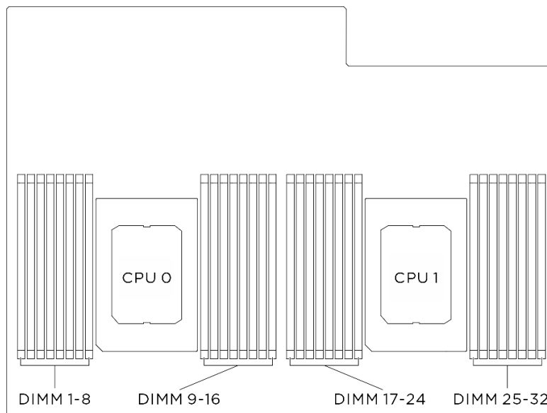
圖例 283. 記憶體模組和處理器佈置
