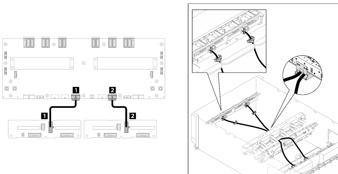
圖例 380. 前方 2.5 吋硬碟背板電源線佈線
