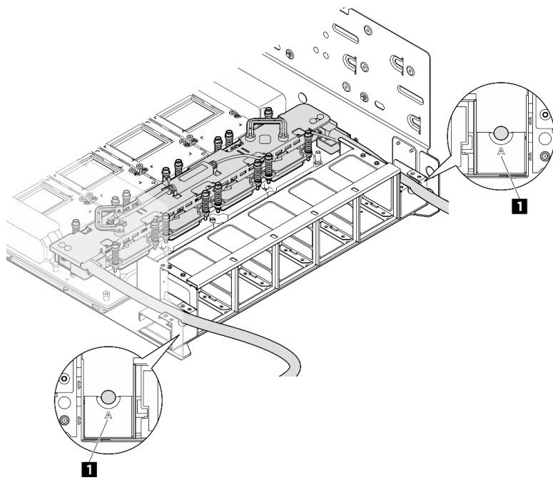
圖例 130. 放置軟管
