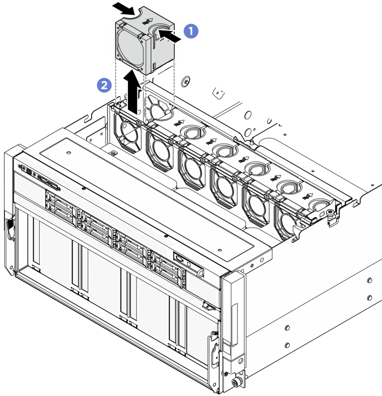
圖例 50. 卸下前方風扇
