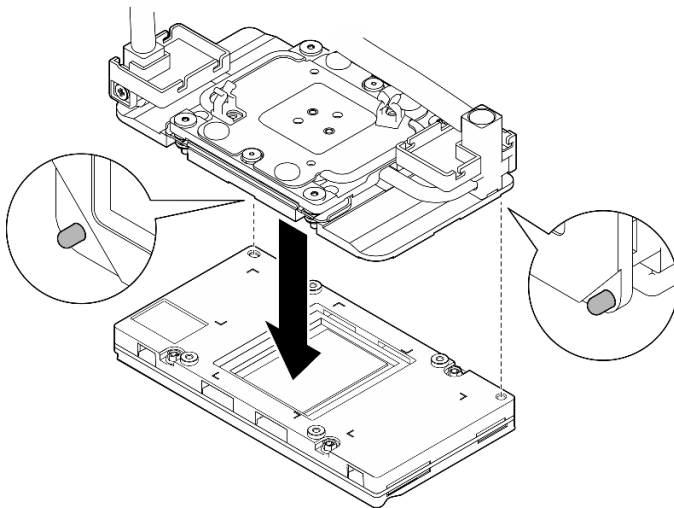
圖例 156. 調整 GPU 水冷板
