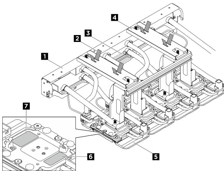
圖例 149. 前方 H100/H200 GPU 水冷板模組元件識別
