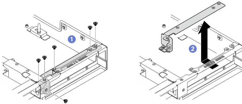
圖例 348. 卸下背面框架支撐托架
