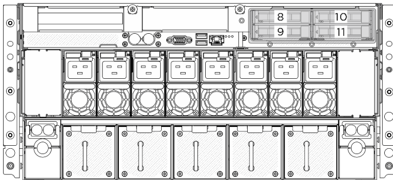
圖例 349. 後方 2.5 吋硬碟背板編號
