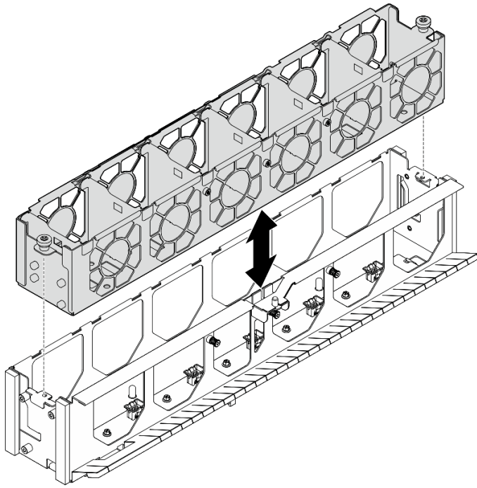
圖例 61. 卸下內部風扇機盒
