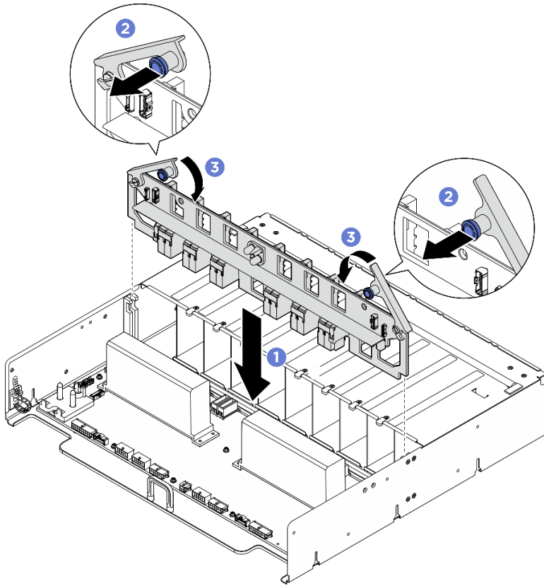
圖例 328. 安裝 PSU 轉插卡
