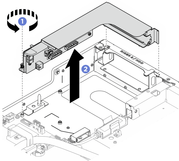
圖例 299. 卸下插槽 2 中的 PCIe 擴充卡組件
