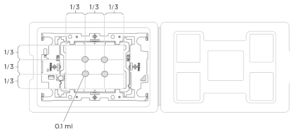
圖例 262. 運送匣中的處理器塗上散熱膏
