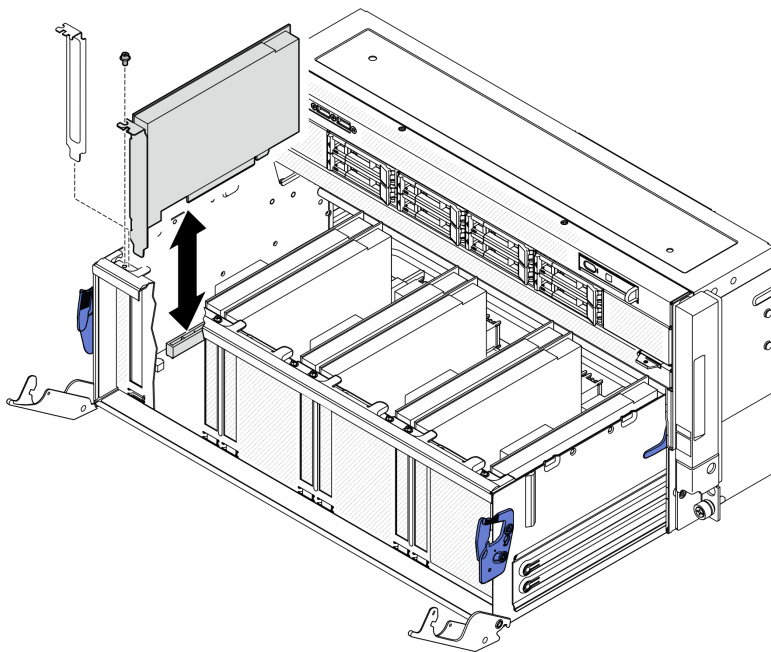
圖例 292. 安裝正面 PCIe 配接卡
