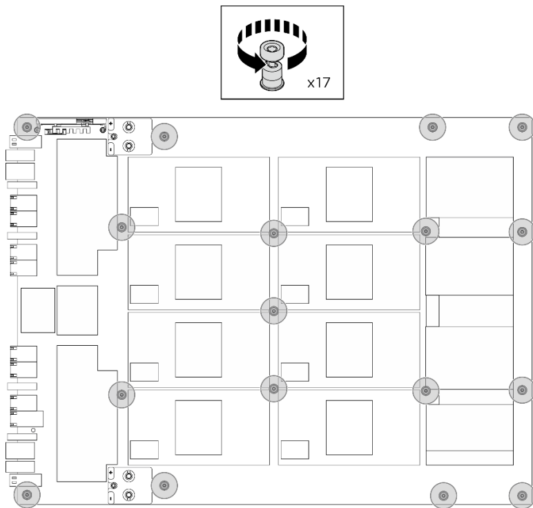
圖例 79. 卸下螺絲
