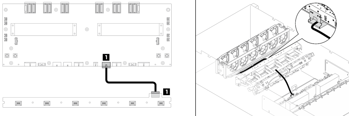
圖例 383. 前方風扇控制板纜線佈線
