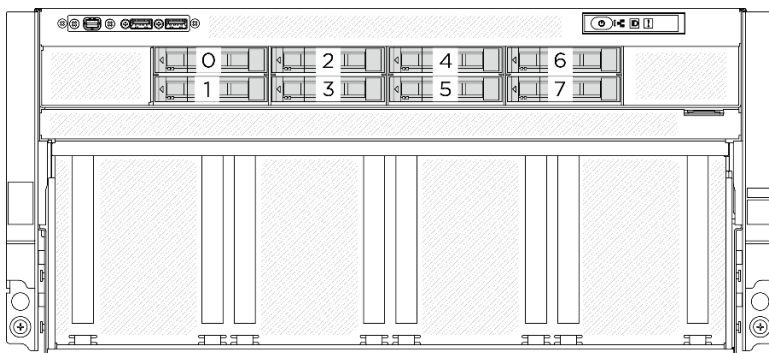
圖例 8. 前方 2.5 吋機槽編號
