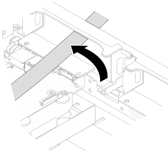
圖例 256. 卸下軟管
