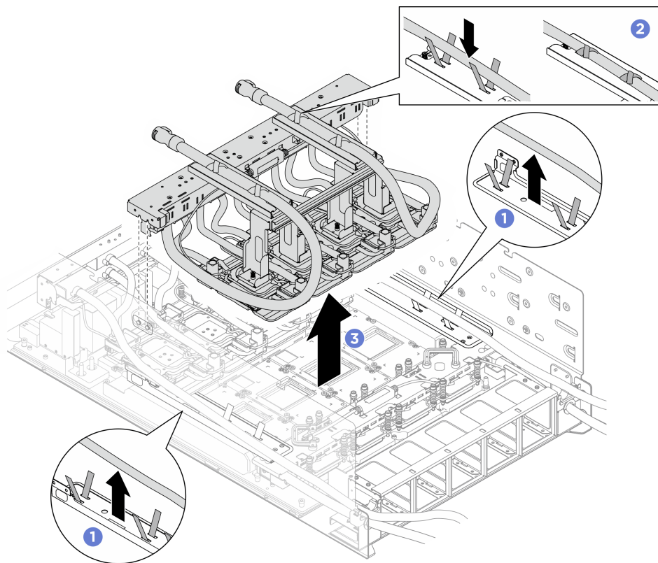
圖例 173. 卸下後方 H100/H200 GPU 水冷板模組
