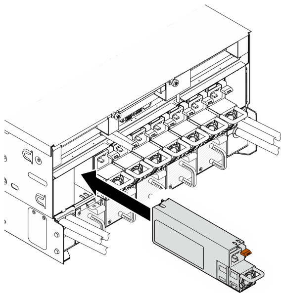
圖例 333. 安裝電源供應器
