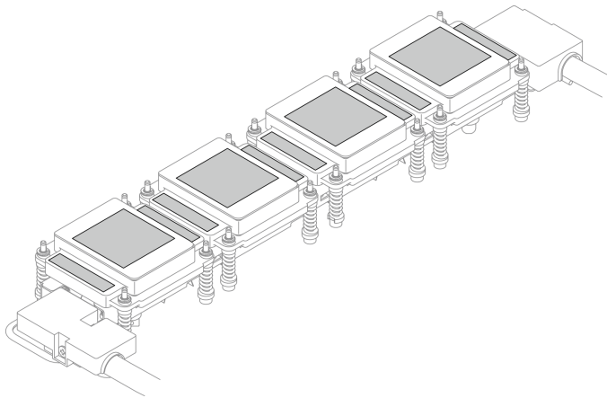
圖例 123. 擦掉水冷板上的 PCM 和油灰墊
