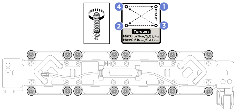
圖例 128. 安裝 NVSwitch 水冷板
