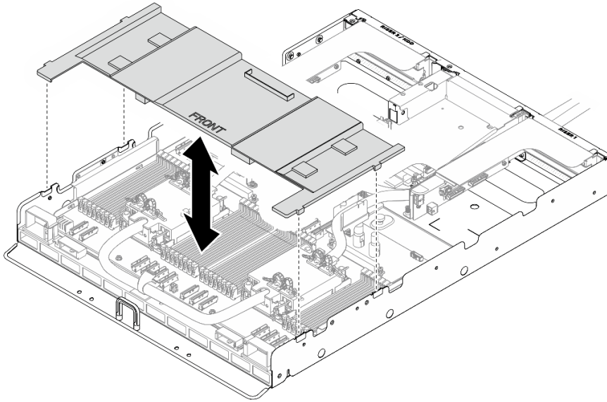
圖例 334. 卸下處理器空氣擋板
