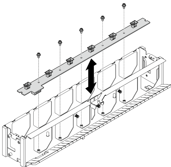
圖例 63. 安裝前方風扇控制板
