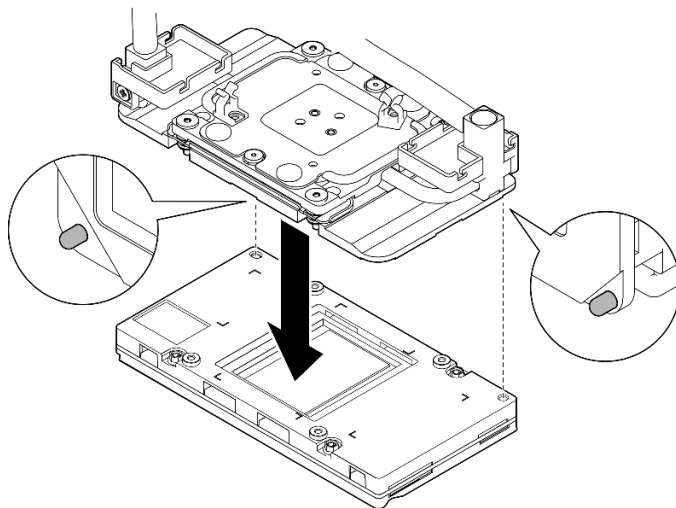
圖例 182. 調整 GPU 水冷板
