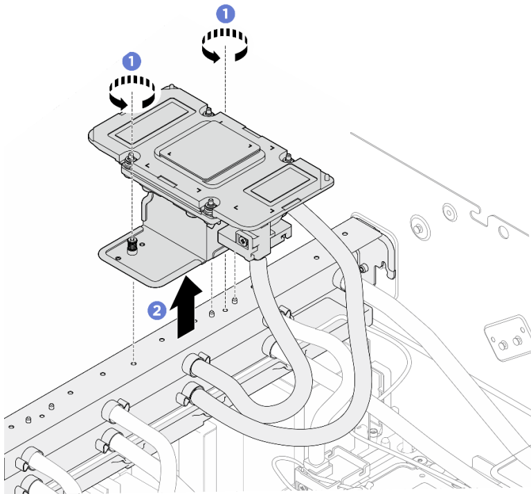
圖例 209. 卸下維修托架和 GPU 水冷板組件
