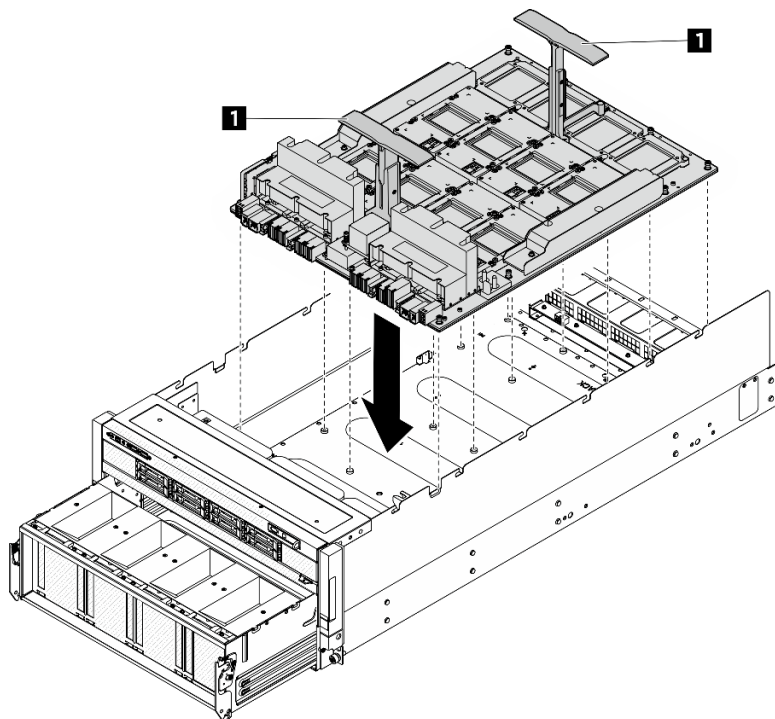
圖例 88. 安裝 GPU 複合體
