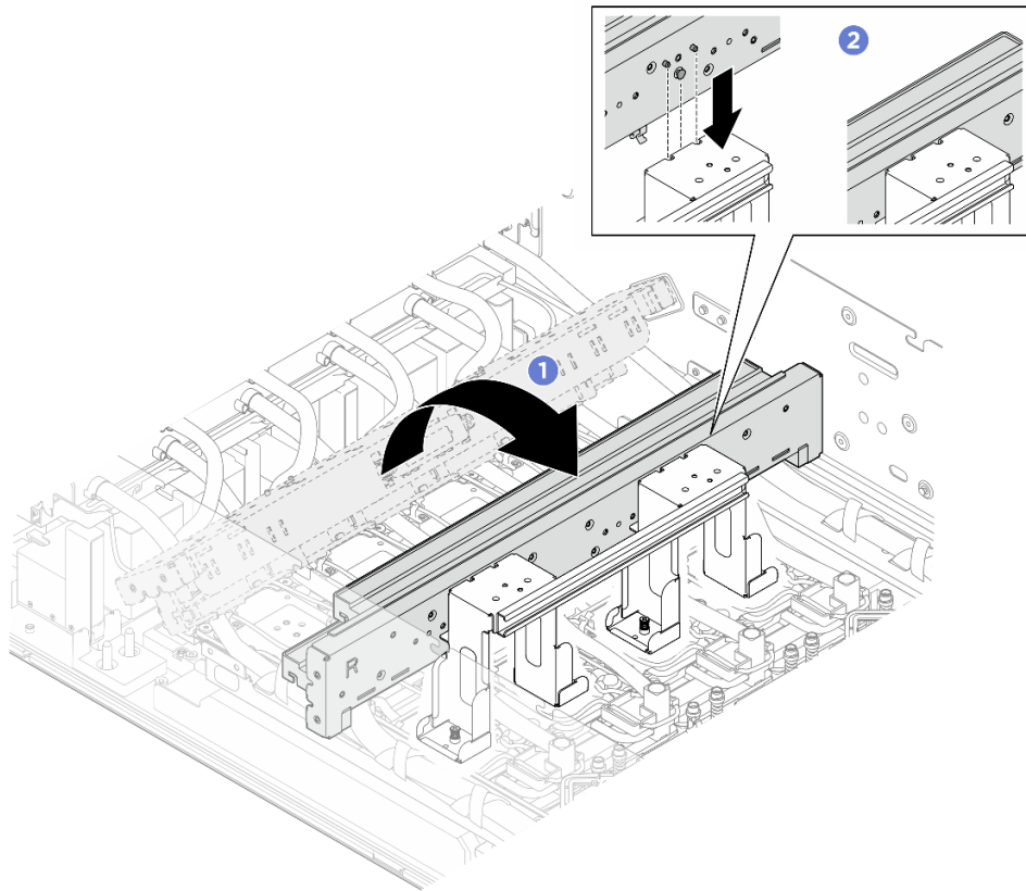
圖例 195. 重新放置後方 GPU 水冷板模組歧管
