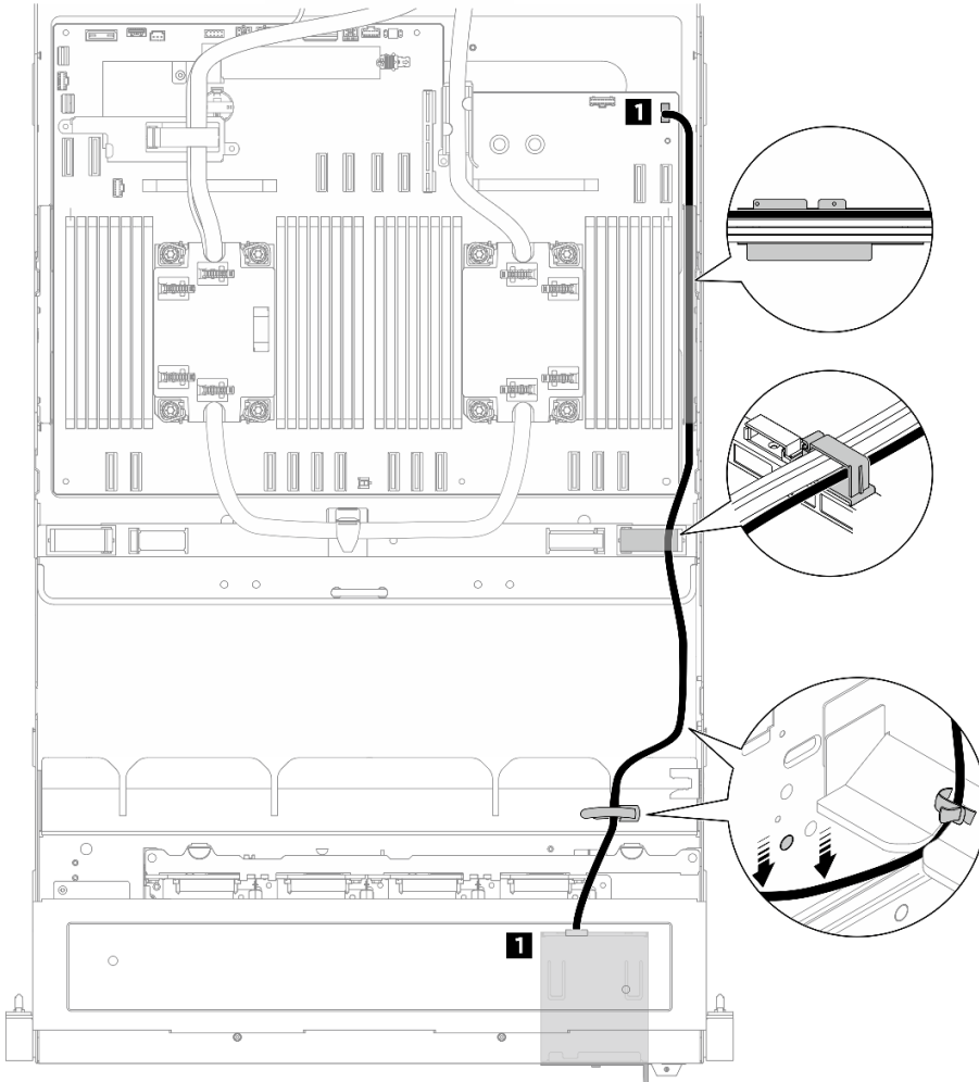
圖例 387. 整合式診斷面板纜線佈線
