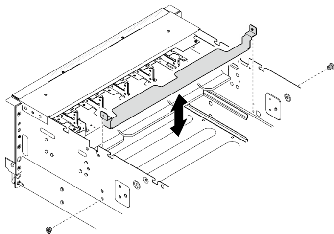
圖例 92. 安裝 GPU 接頭保護托架
