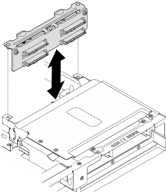
圖例 350. 卸下後方 2.5 吋硬碟背板托架
