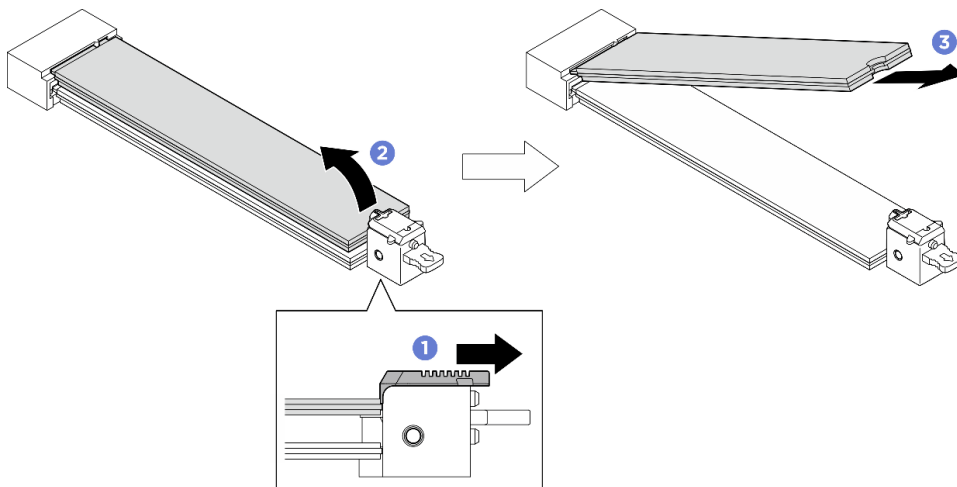
圖例 278. 卸下上方 M.2 硬碟
