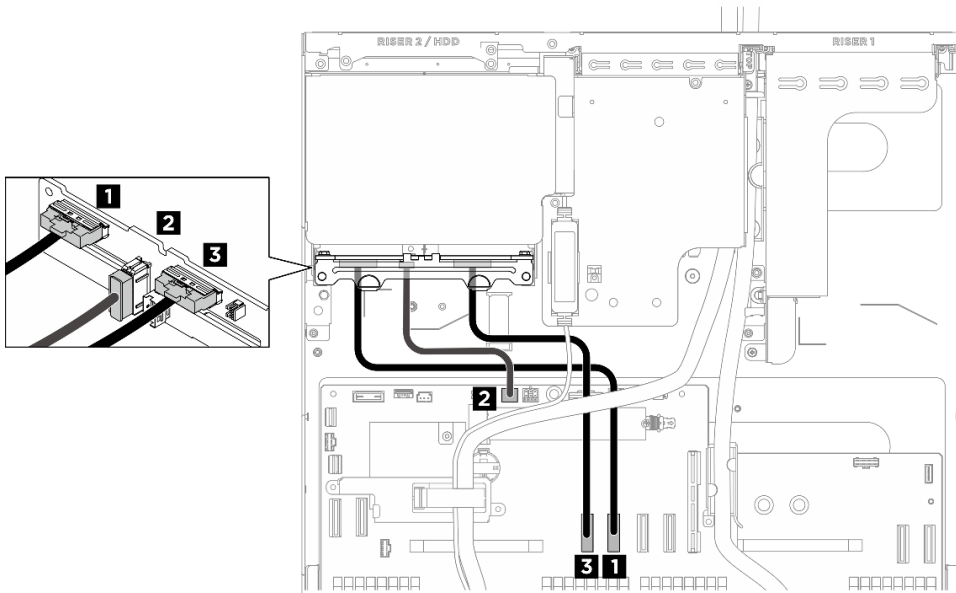
圖例 381. 後方 2.5 吋硬碟背板纜線佈線
