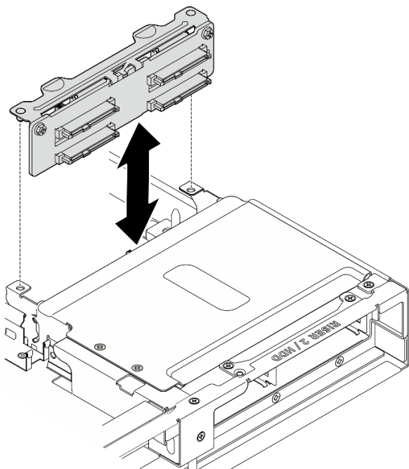
圖例 354. 安裝後方 2.5 吋硬碟背板托架
