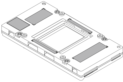
圖例 225. 清除 GPU 上的 PCM 和油灰墊
