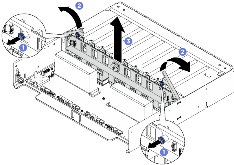
圖例 337. 卸下 PSU 轉插卡
