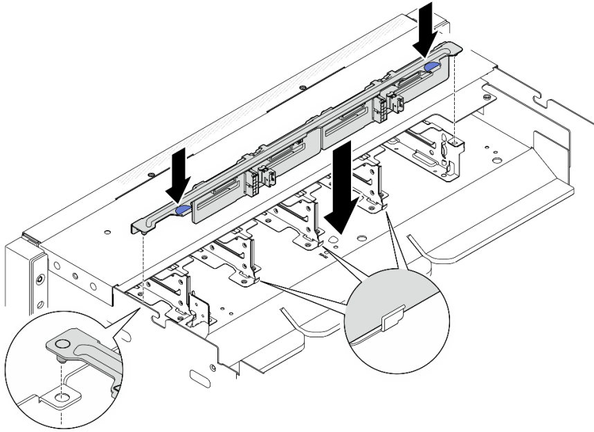
圖例 21. 安裝前方 2.5 吋硬碟背板托架
