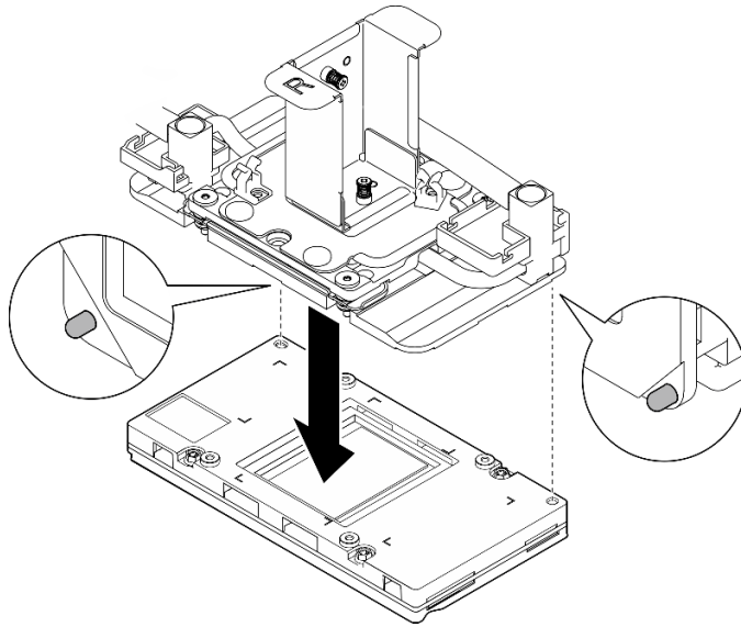
圖例 234. 調整水冷板
