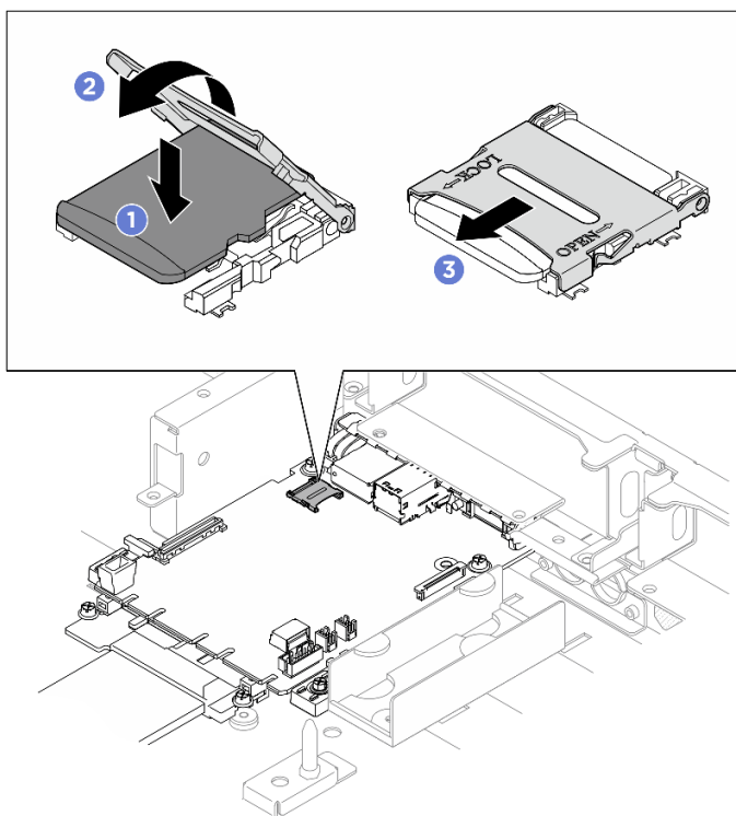
圖例 288. 安裝 MicroSD 卡
