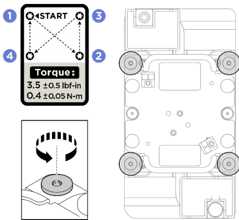
圖例 221. 卸下 GPU 水冷板
