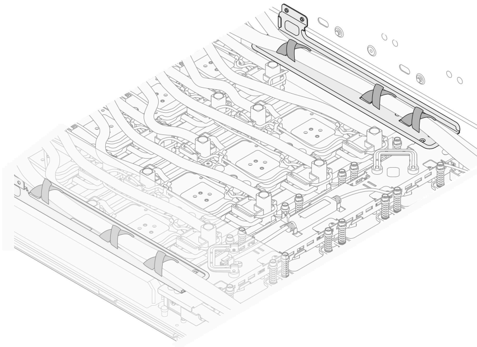
圖例 160. 用軟管束帶固定軟管和纜線
