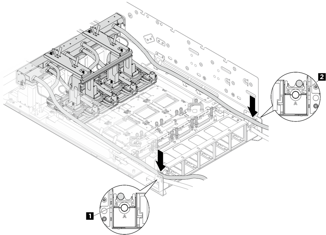
圖例 161. 將軟管放在水管固定器上
