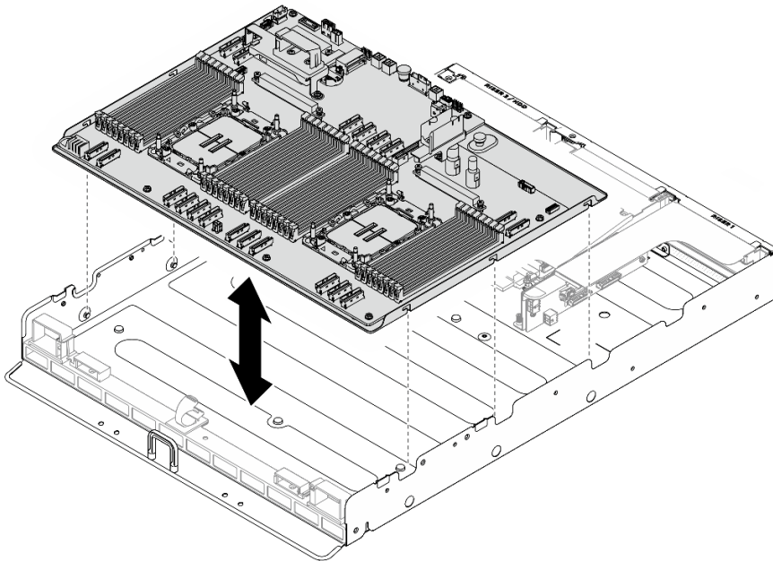
圖例 364. 安裝主機板
