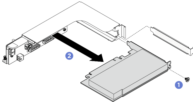
圖例 295. 卸下背面 PCIe 配接卡
