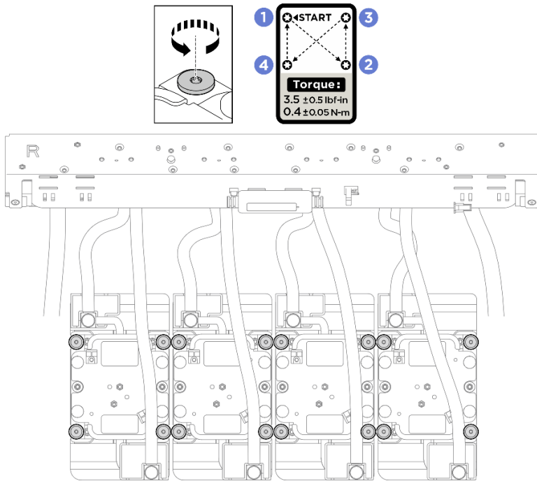
圖例 169. 卸下 GPU 水冷板
