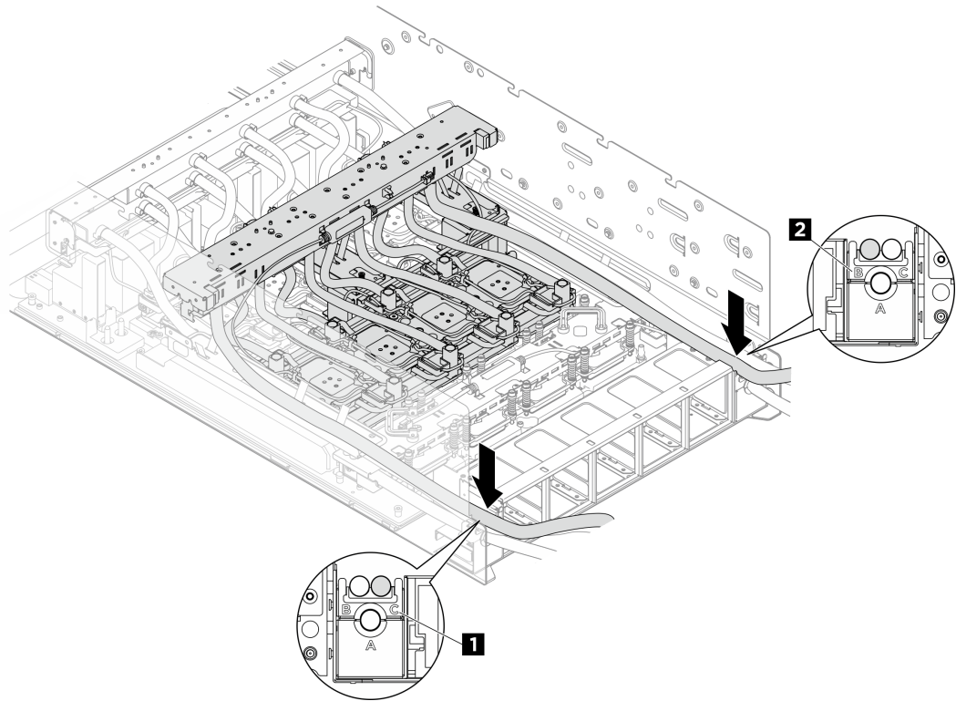
圖例 187. 將軟管放在水管固定器上
