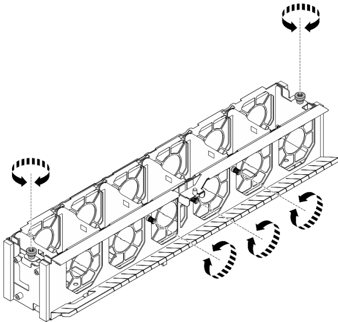
圖例 65. 固定內部風扇機盒
