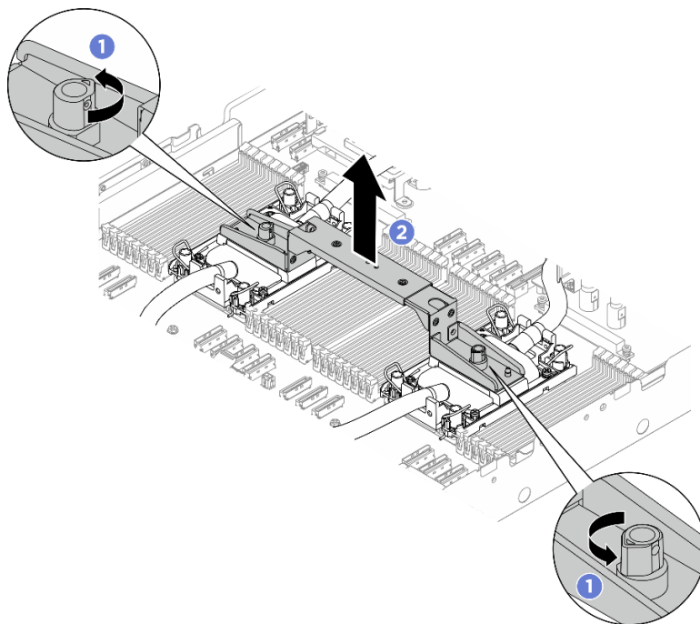
圖例 266. 卸下模組把手
