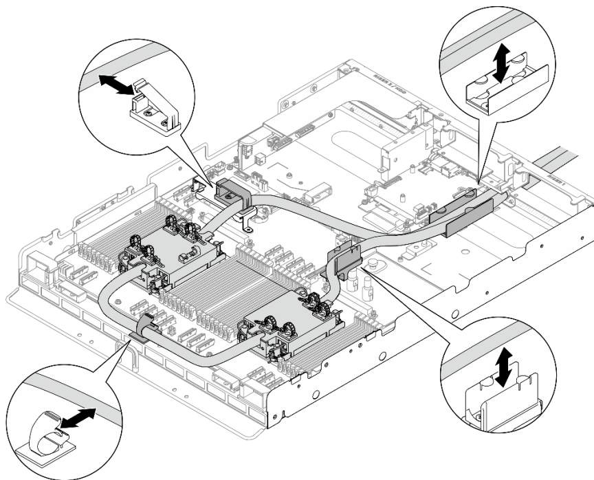
圖例 253. 拔開軟管
