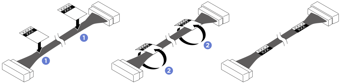
圖例 307. 黏貼標籤
