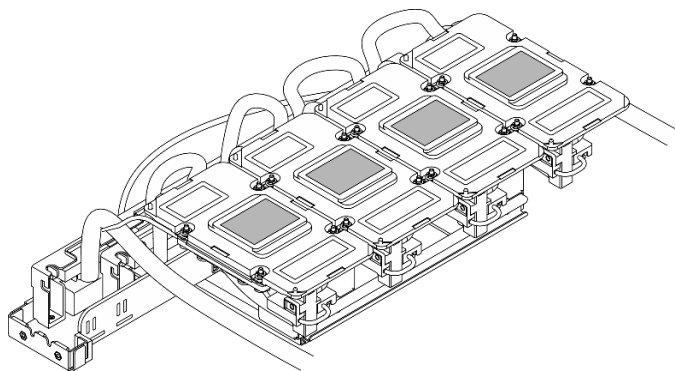
圖例 175. 擦掉水冷板上的 PCM 和油灰墊
