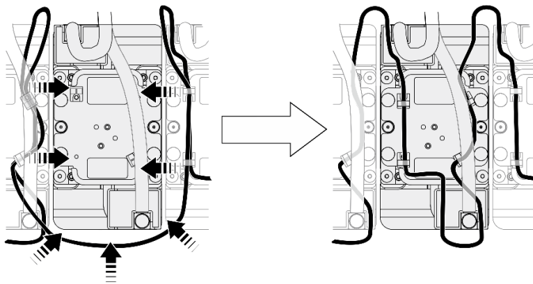
圖例 214. 安裝洩漏感應器模組纜線
