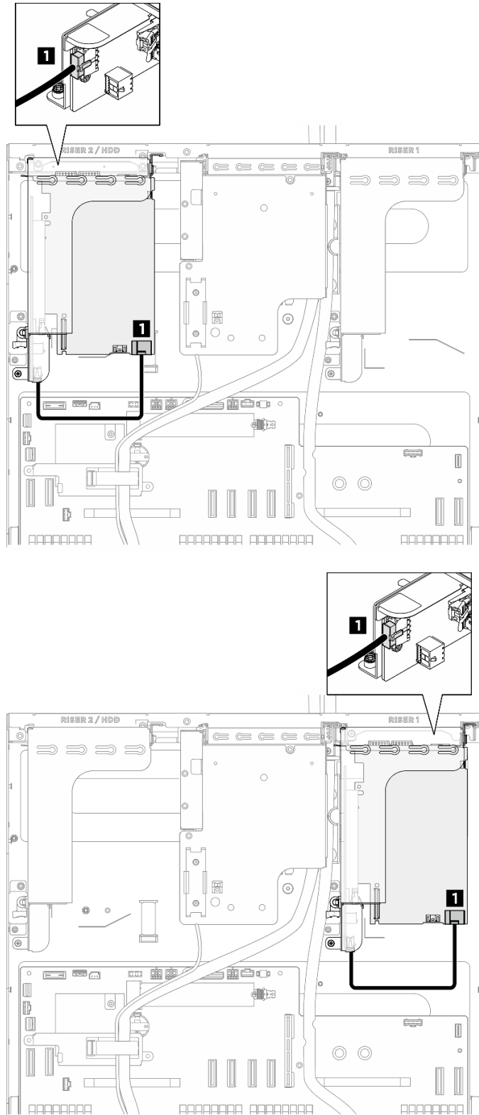
圖例 396. DPU 電源線佈線
