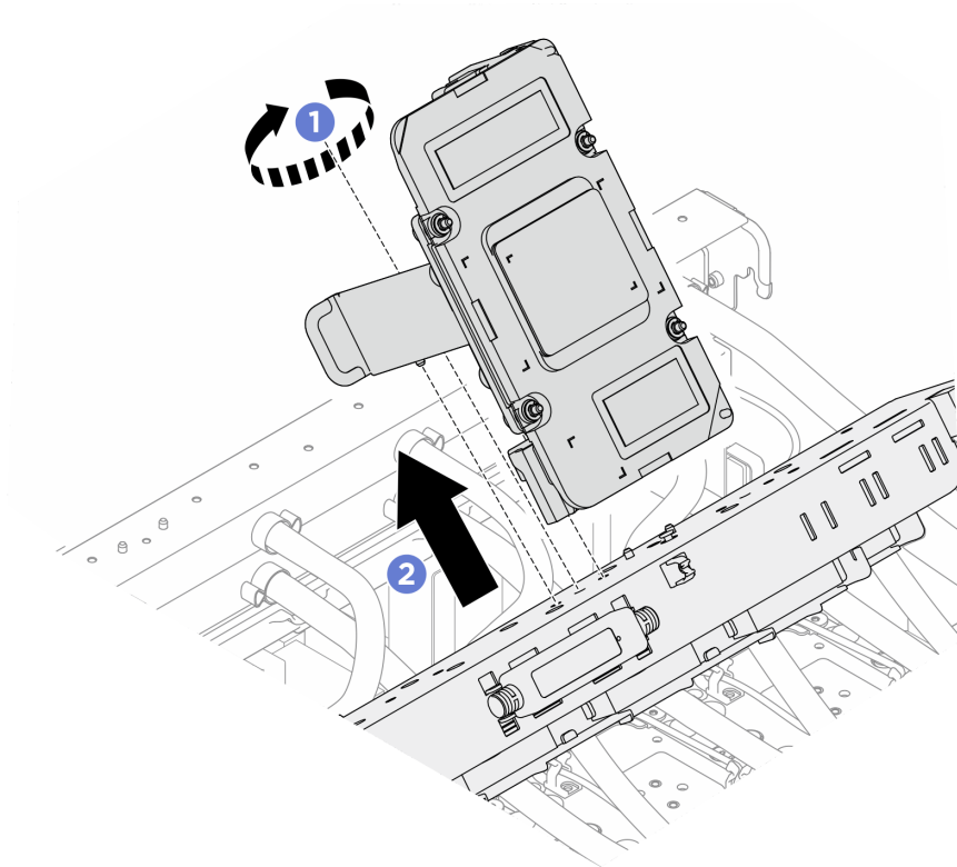
圖例 233. 卸下維修托架和 GPU 水冷板組件
