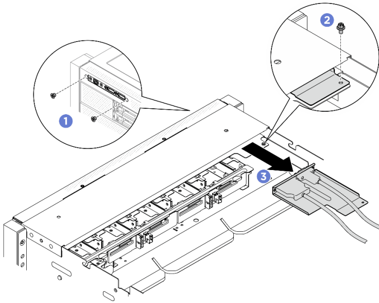
圖例 71. 卸下正面 I/O 模組
