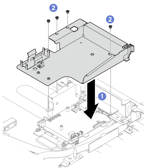
圖例 274. 安裝洩漏感應器模組匣托架
