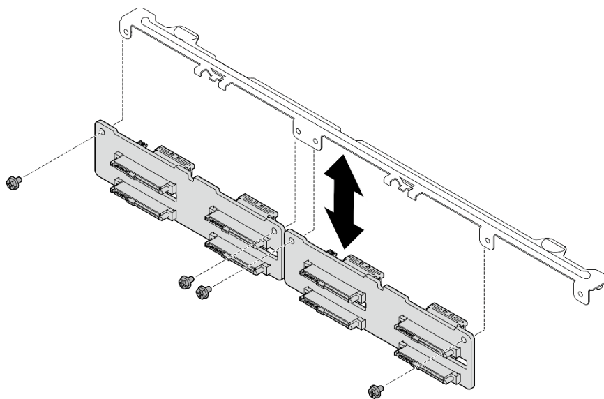
圖例 20. 安裝前方 2.5 吋硬碟背板
