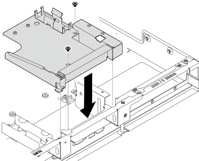
圖例 357. 安裝洩漏感應器模組托架
