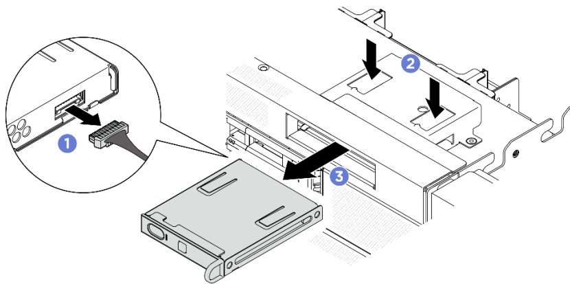
圖例 241. 卸下整合式診斷面板
