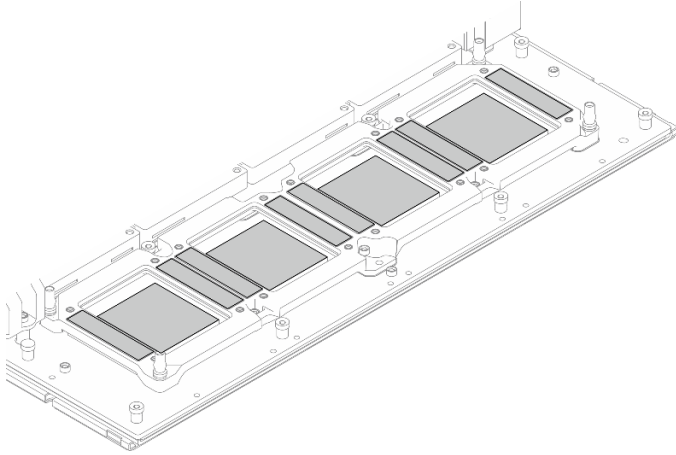
圖例 122. 清除 NVSwitch 上的 PCM 和油灰墊
