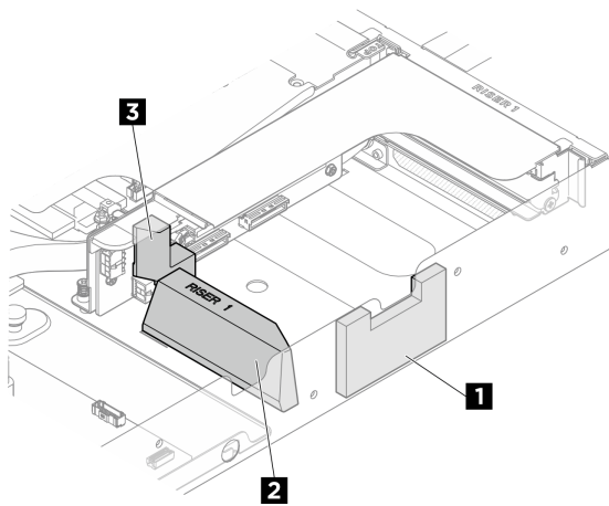
圖例 38. DPU 空氣擋板在擴充卡 1 插槽中的位置
