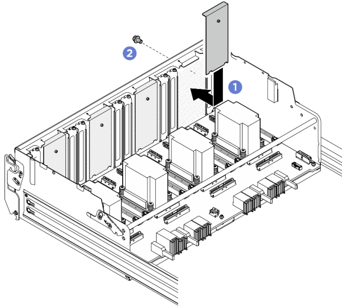
圖例 370. 安裝排氣區塊
