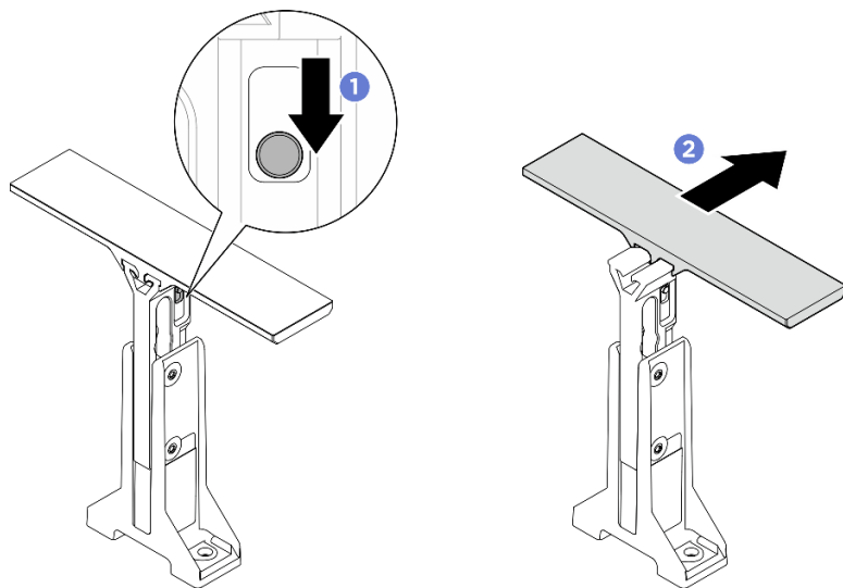
圖例 89. 調整把手
