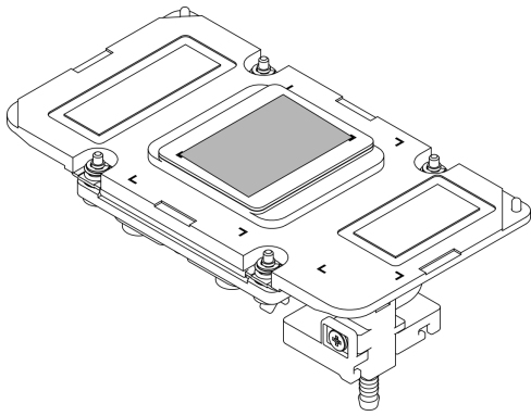
圖例 226. 擦掉水冷板上的 PCM 和油灰墊
