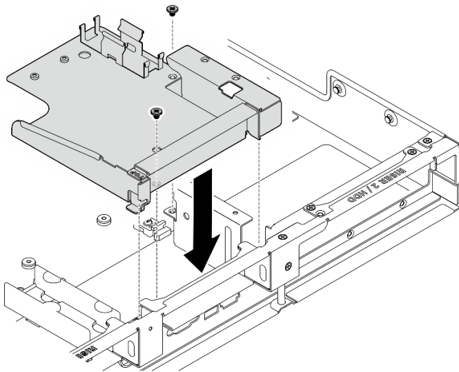
圖例 249. 安裝洩漏感應器模組托架
