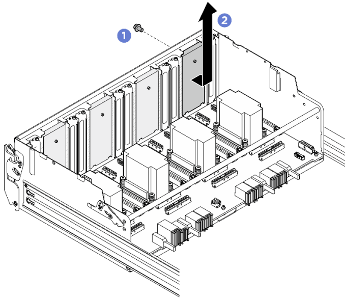
圖例 369. 卸下排氣區塊
