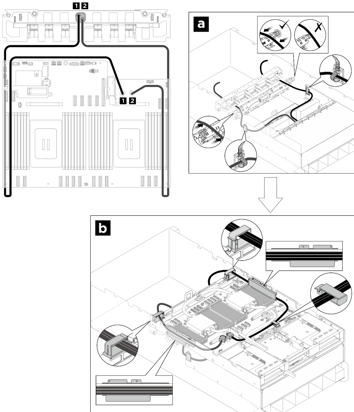
圖例 394. PSU 轉插卡至主機板纜線佈線
