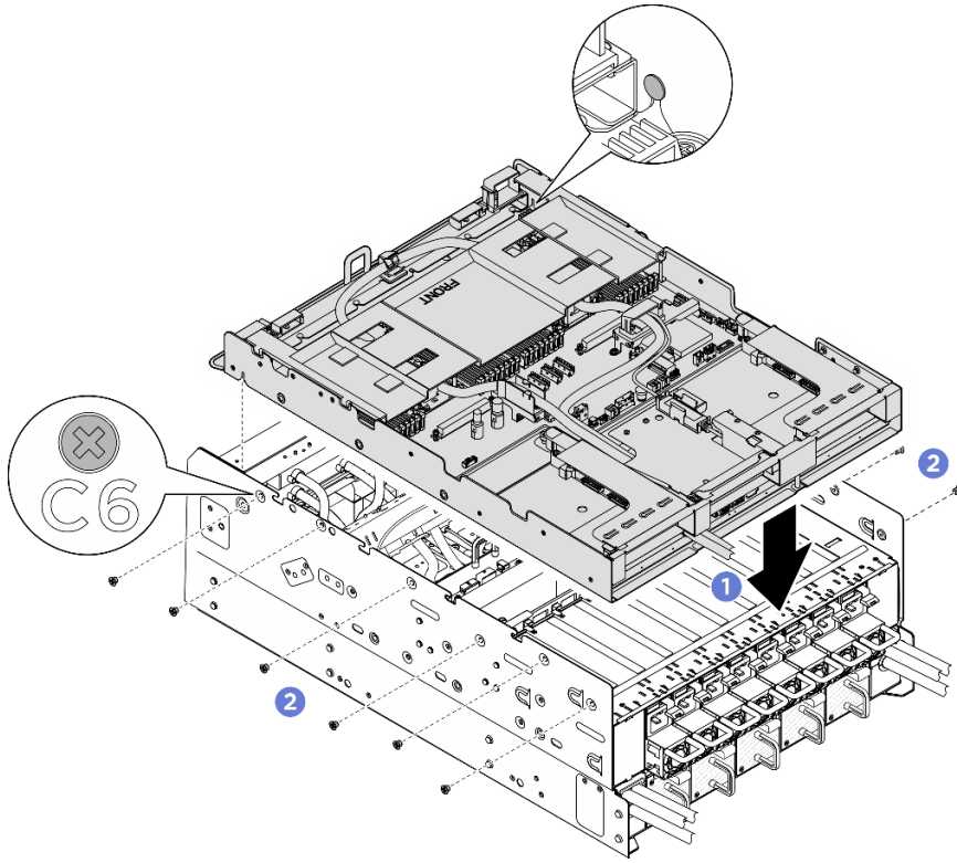
圖例 24. 安裝 CPU 複合體
