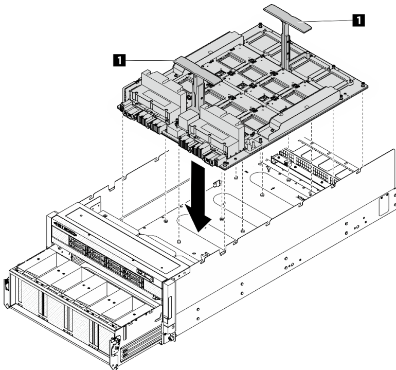
圖例 101. 安裝 GPU 複合體
