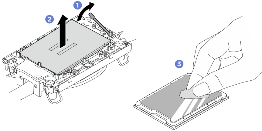
圖例 259. 卸下處理器
