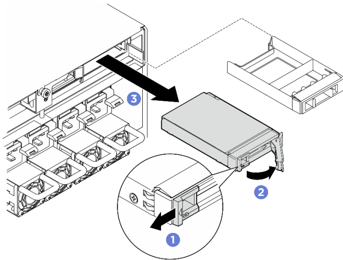
圖例 11. 卸下後方 2.5 吋熱抽換硬碟
