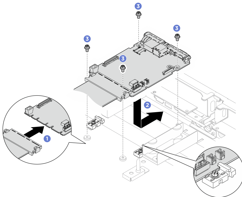
圖例 360. 安裝系統 I/O 板
