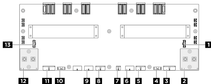
圖例 376. 電源配送板接頭
