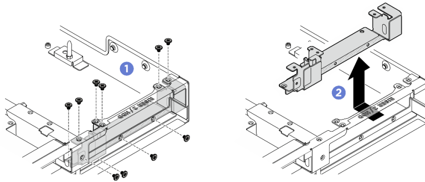
圖例 300. 卸下背面擴充卡支撐托架
