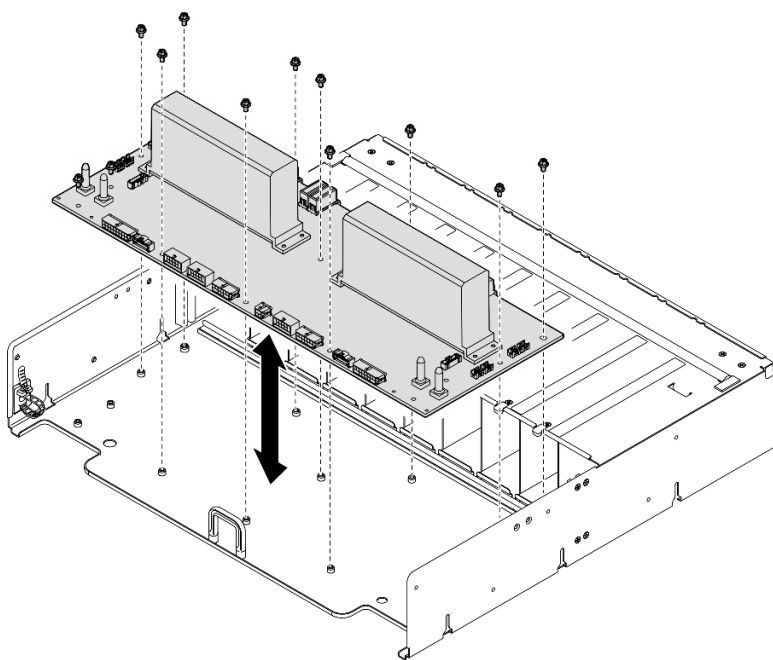
圖例 325. 卸下電源配送板
