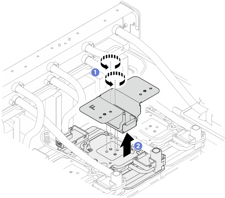
圖例 211. 卸下維修托架
