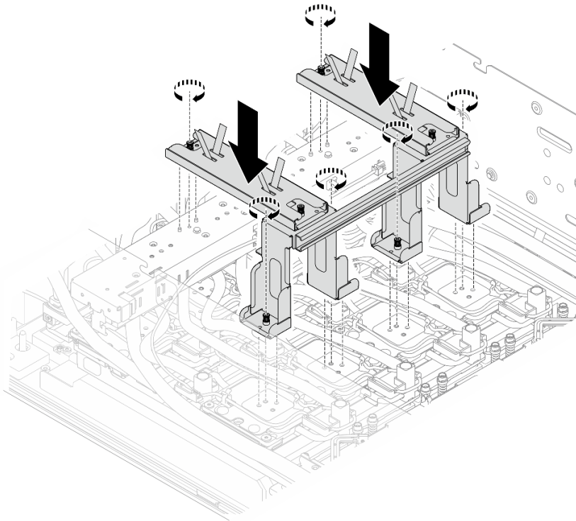
圖例 172. 安裝出貨托架
