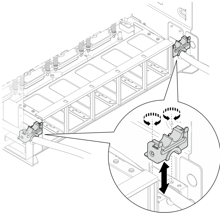
圖例 116. 卸下水管固定器 B/C
