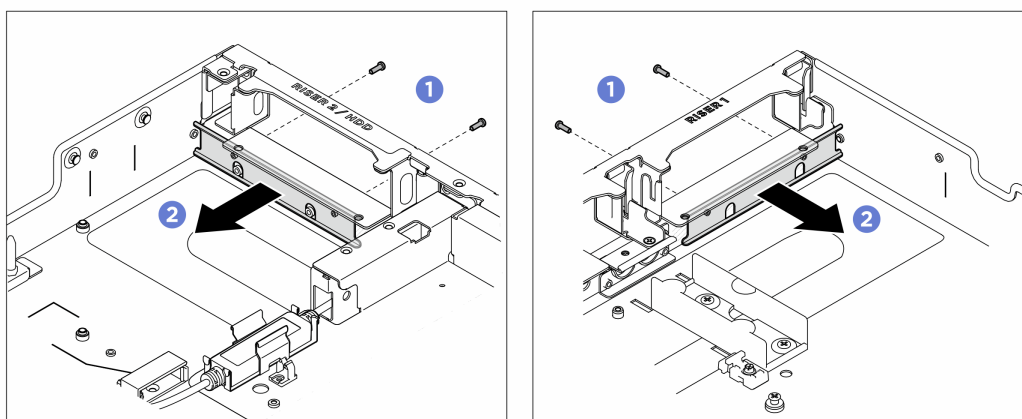
圖例 367. 卸下排氣區塊
