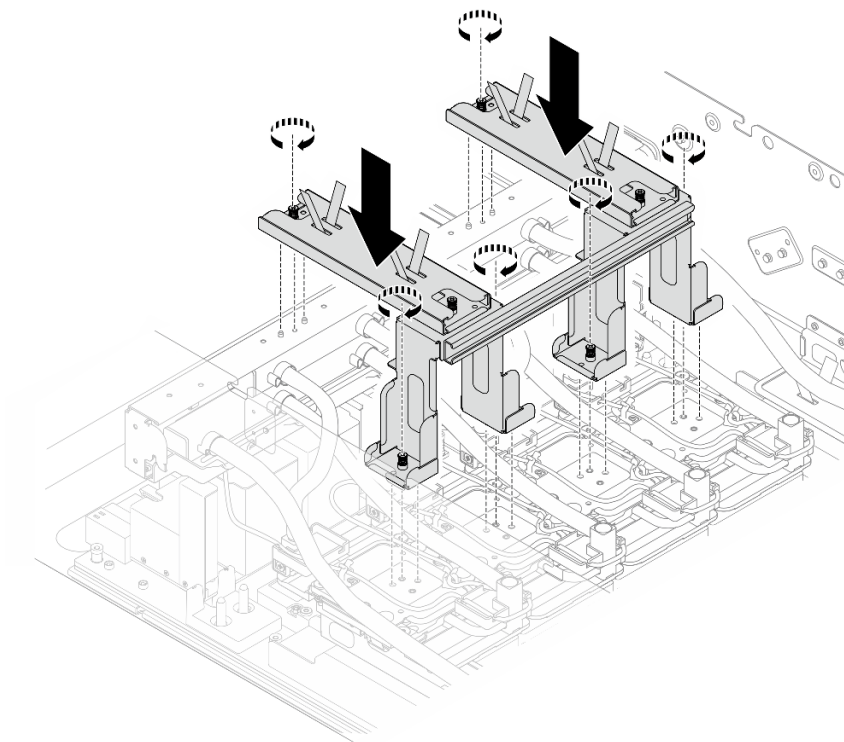
圖例 142. 安裝出貨托架
