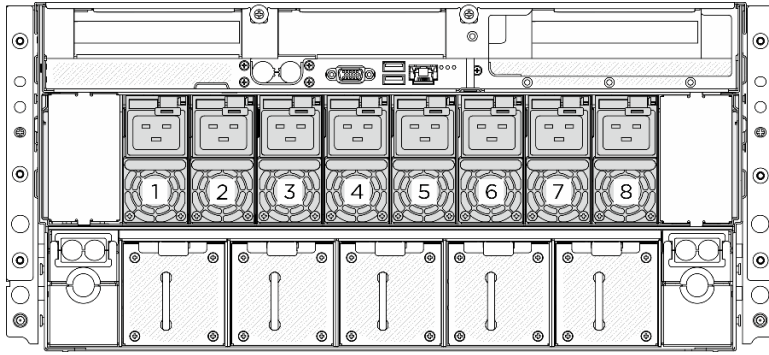
圖例 332. 電源供應器機槽編號
