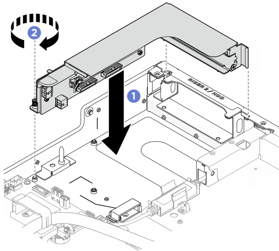
圖例 306. 將 PCIe 擴充卡組件安裝在插槽 2 中
