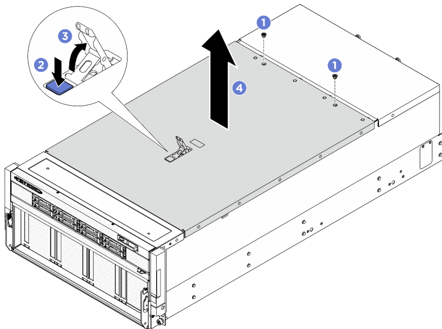
圖例 4. 卸下前方上蓋
