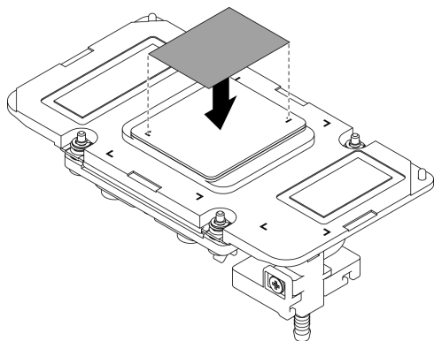
圖例 207. 貼附 PCM
