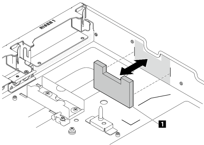
圖例 40. 將擴充卡插槽 1 DPU 空氣擋板安裝到機箱
