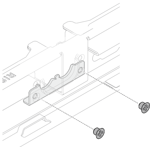
圖例 254. 卸下水管固定器
