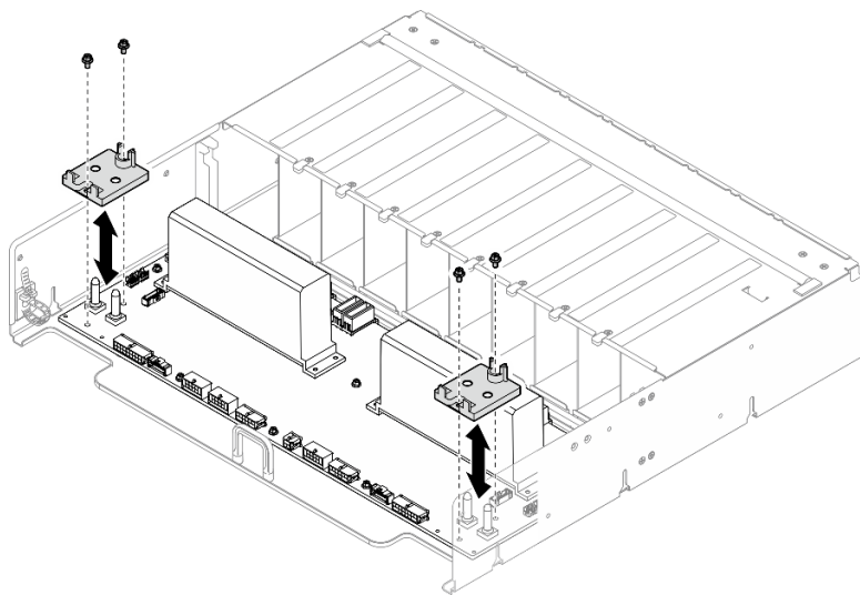
圖例 324. 卸下纜線固定器
