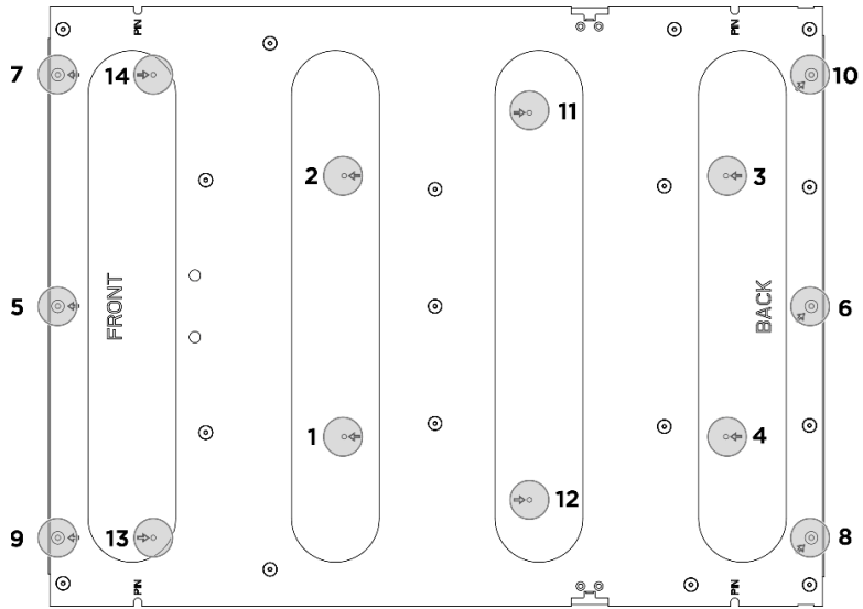
圖例 109. GPU 複合體配接器板螺絲順序
