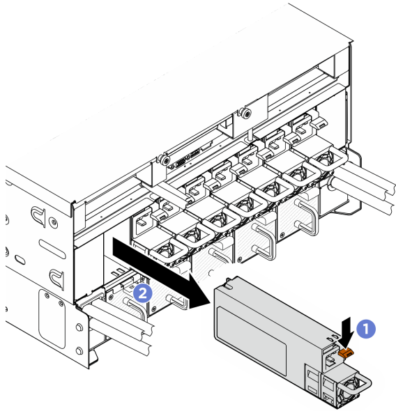
圖例 331. 電源供應器卸下
