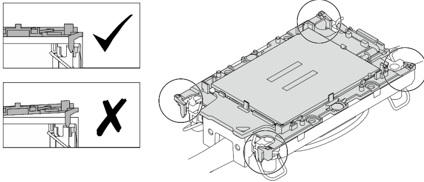
圖例 264. 檢查處理器與水冷板
