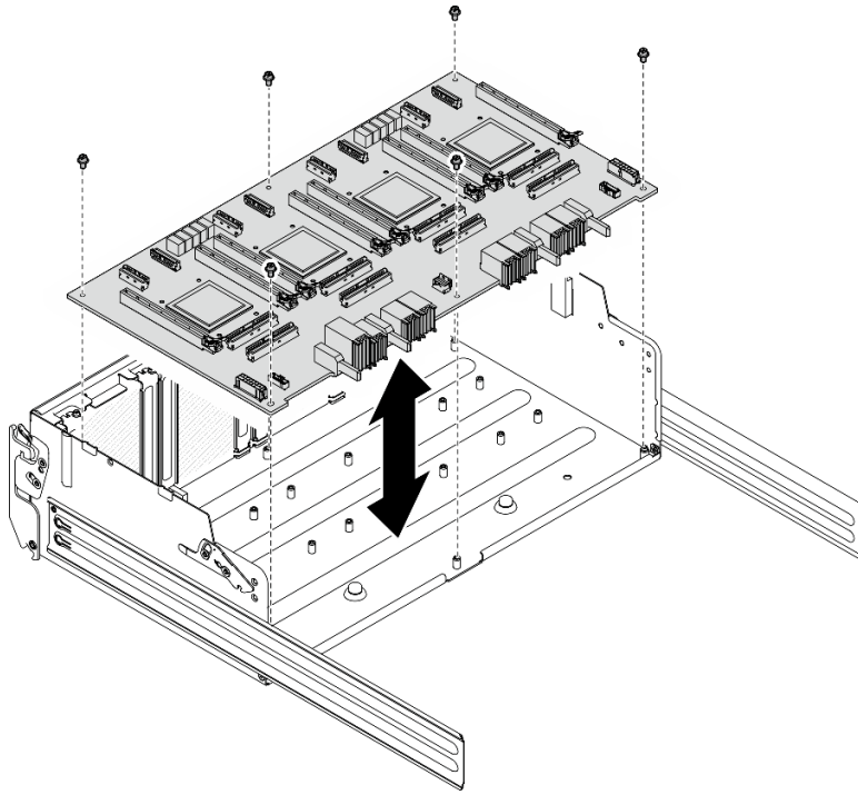
圖例 309. 卸下 PCIe 交換器板
