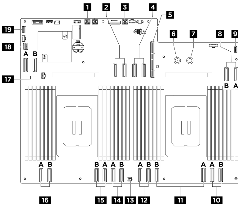
圖例 378. 用於纜線佈線的主機板接頭
