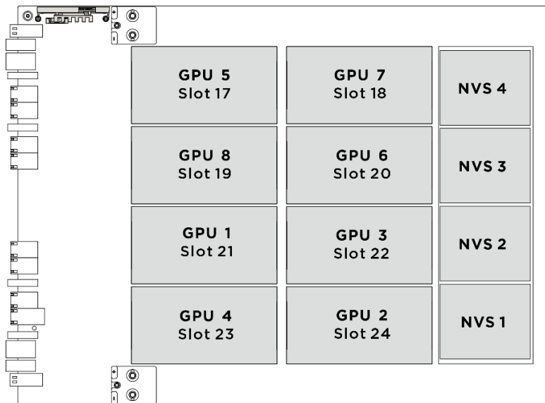
圖例 148. GPU 編號
