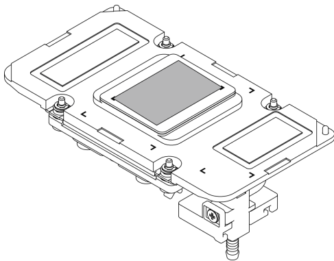
圖例 202. 擦掉水冷板上的 PCM 和油灰墊
