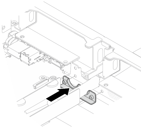
圖例 270. 安裝水管固定器
