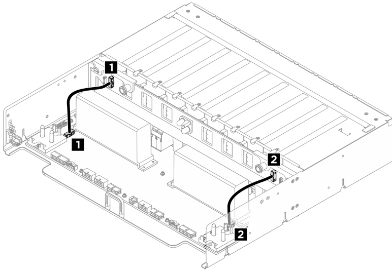
圖例 393. PSU 轉插卡到電源配送板纜線佈線
