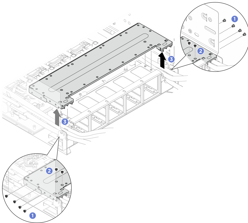
圖例 115. 卸下後方風扇機盒支撐托架
