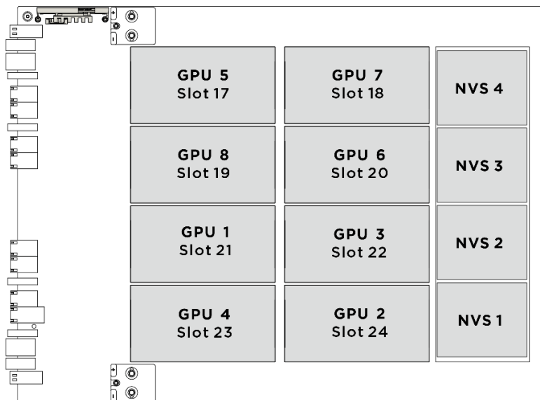
圖例 228. GPU 編號
