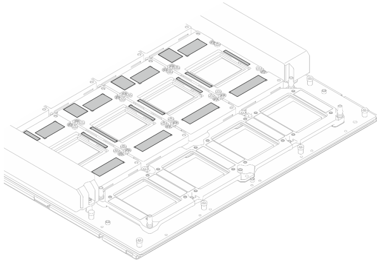
圖例 174. 清除 GPU 上的 PCM 和油灰墊
