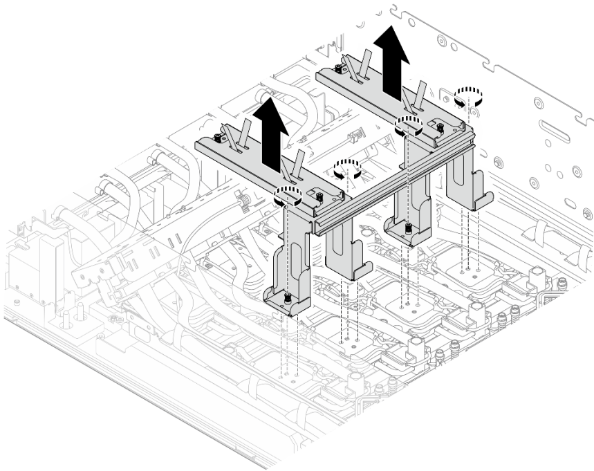
圖例 218. 卸下出貨托架
