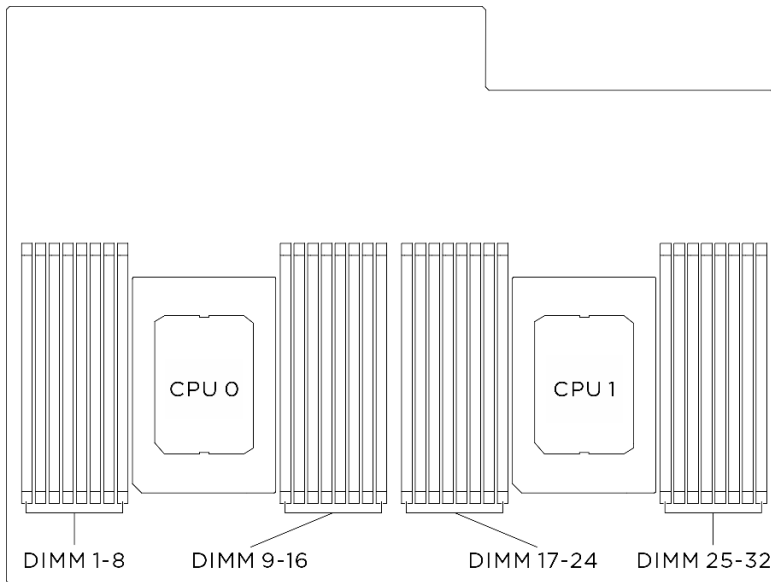
圖例 285. 記憶體模組和處理器佈置
