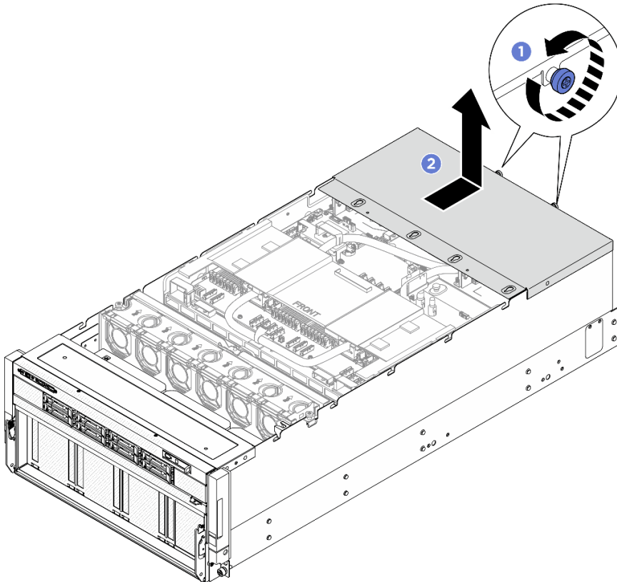
圖例 6. 卸下後方上蓋
