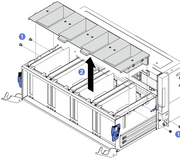
圖例 290. 卸下空氣擋板
