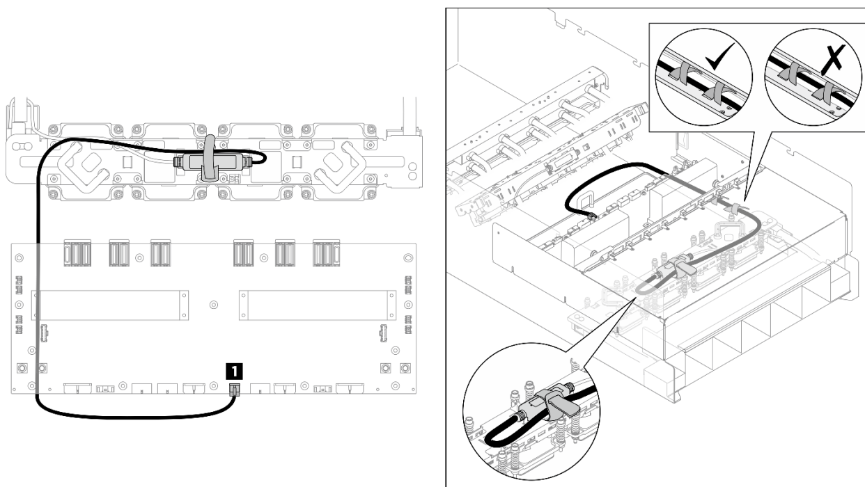
圖例 397. NVSwitch 洩漏感應器模組纜線佈線
