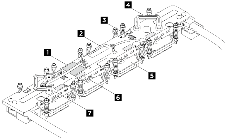
圖例 113. NVSwitch 水冷板模組元件識別
