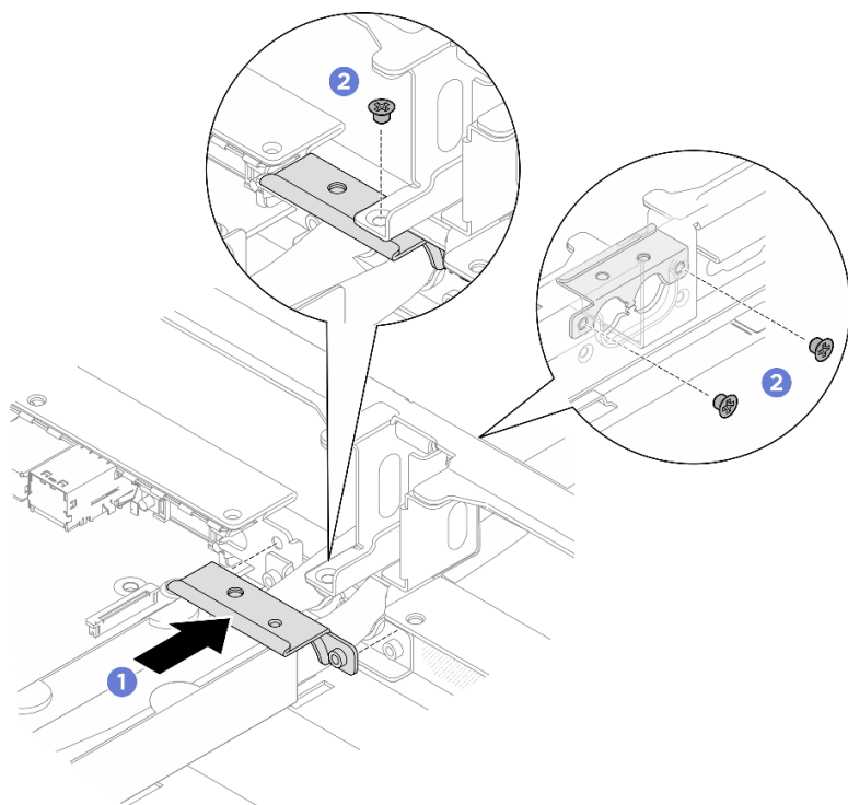
圖例 273. 安裝軟管蓋
