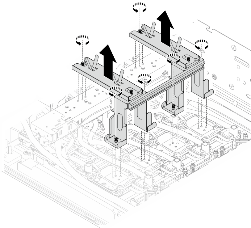
圖例 181. 卸下出貨托架
