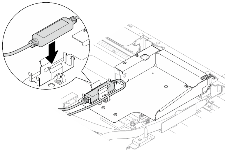
圖例 275. 安裝洩漏感應器模組
