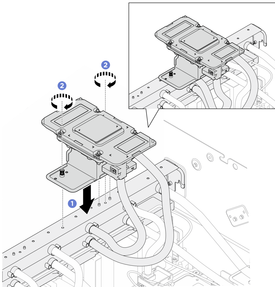
圖例 199. 安裝維修托架和 GPU 水冷板組件
