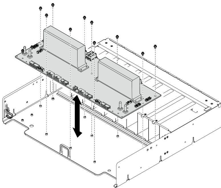
圖例 326. 安裝電源配送板
