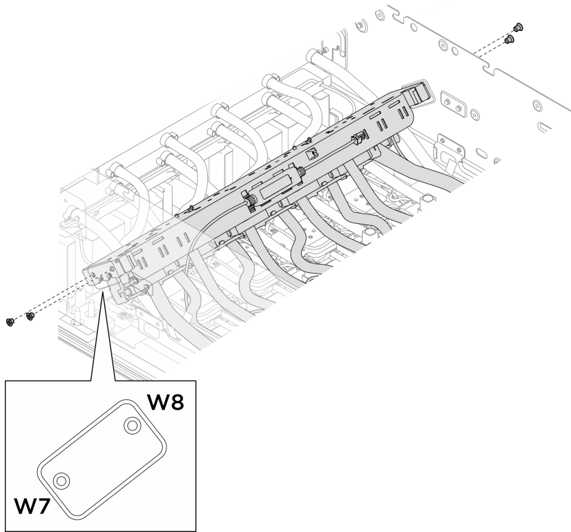
圖例 194. 卸下後方 H100/H200 GPU 水冷板模組歧管
