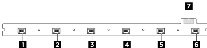
圖例 372. 前方風扇控制板接頭
