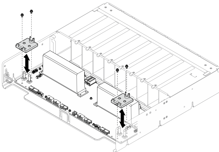
圖例 341. 安裝纜線固定器
