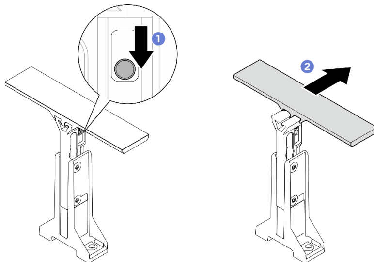
圖例 102. 調整把手
