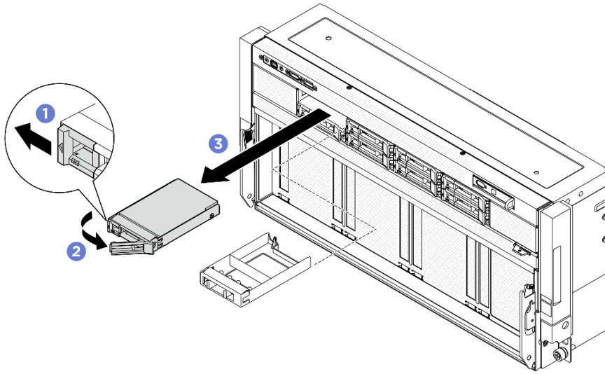
圖例 10. 卸下前方 2.5 吋熱抽換硬碟
