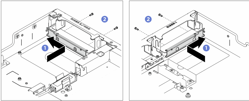
圖例 368. 安裝排氣區塊
