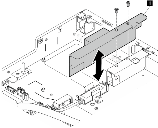
圖例 34. 卸下 DPU 空氣擋板和托架組件
