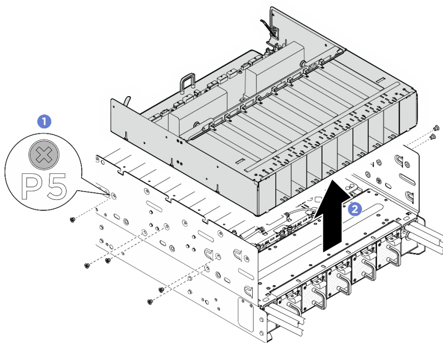
圖例 336. 卸下電源複合體
