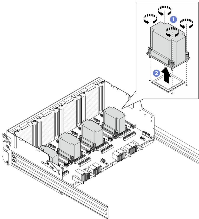
圖例 308. 卸下 PCIe 交換器板散熱槽
