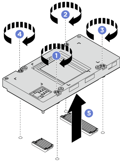
圖例 203. 卸下 GPU
