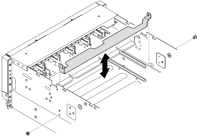
圖例 78. 卸下 GPU 接頭保護托架
