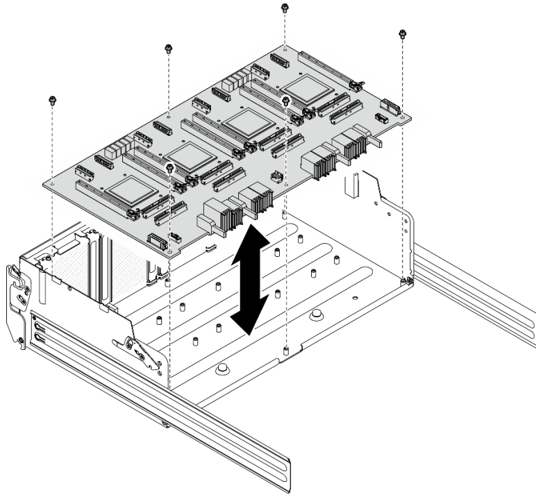
圖例 310. 安裝 PCIe 交換器板
