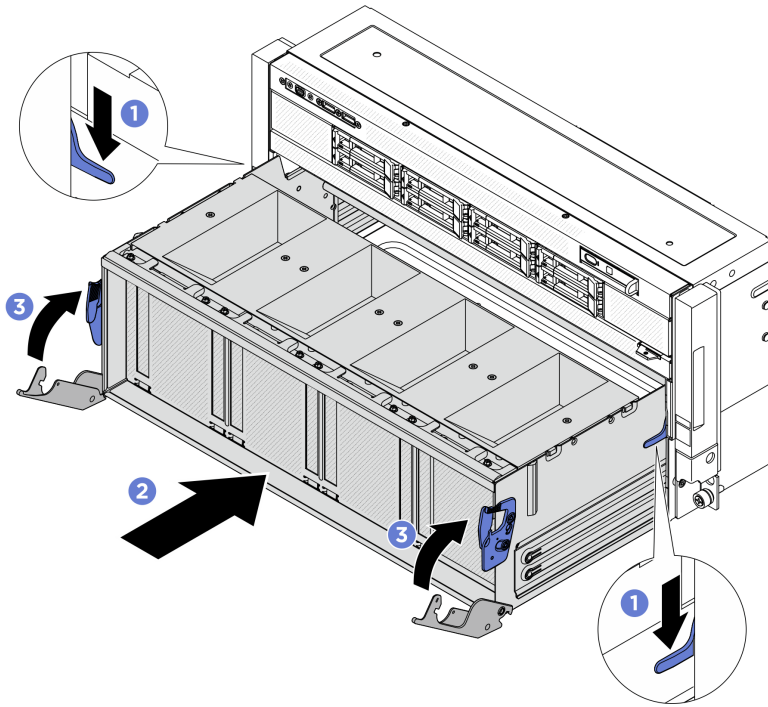
圖例 319. 安裝 PCIe 交換器滑動箱
