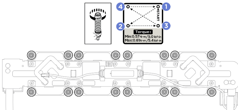
圖例 120. 卸下 NVSwitch 水冷板
