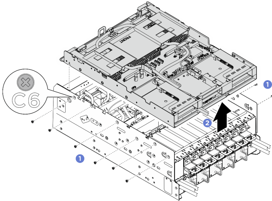
圖例 23. 卸下 CPU 複合體
