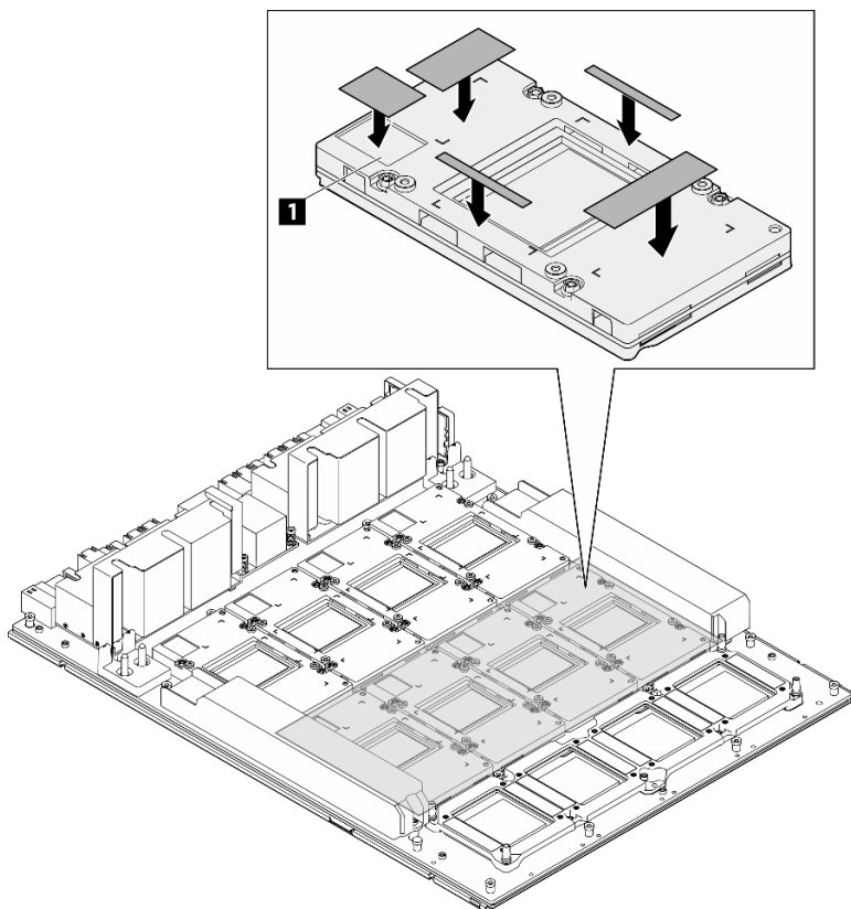
圖例 179. 更換 GPU 油灰墊
