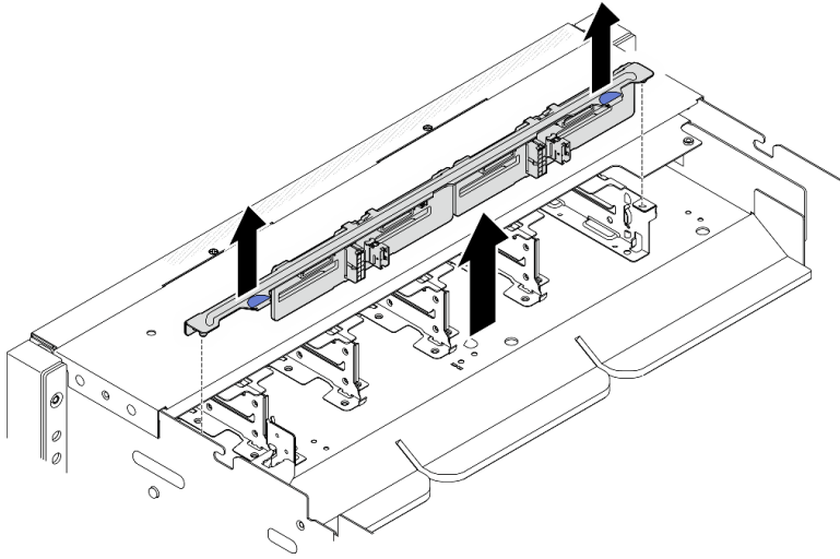
圖例 17. 卸下前方 2.5 吋硬碟背板托架
