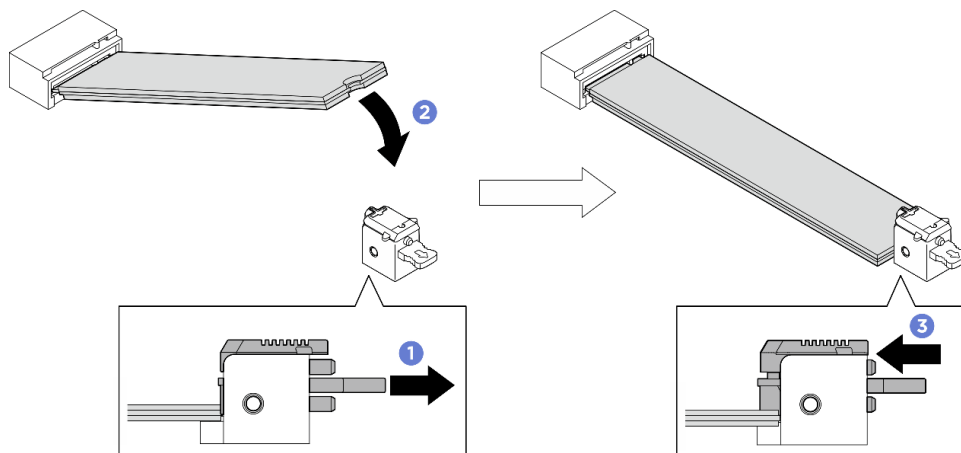
圖例 281. 安裝下方 M.2 硬碟
