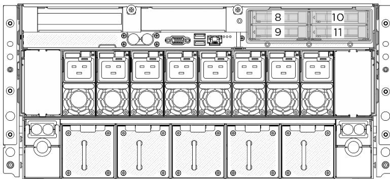
圖例 9. 後方 2.5 吋機槽編號
