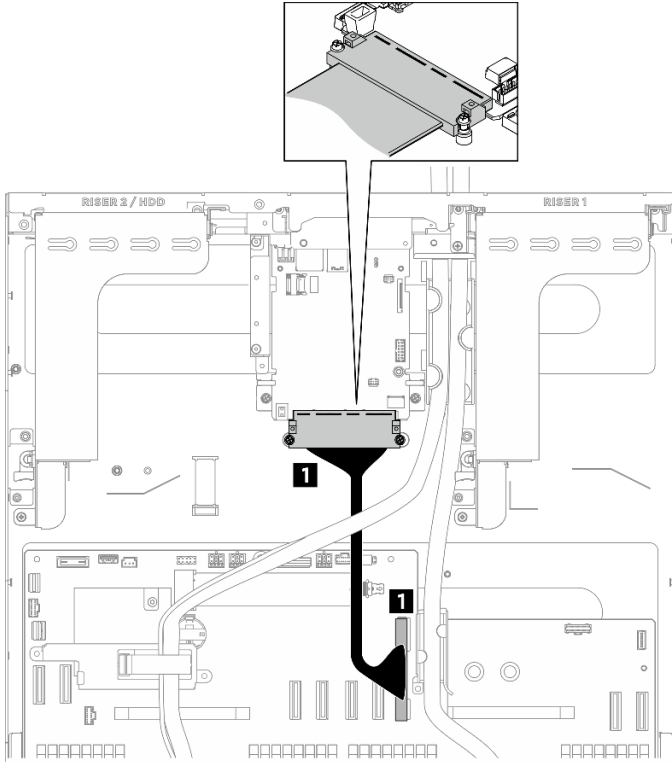
圖例 389. 系統 I/O 板纜線佈線
