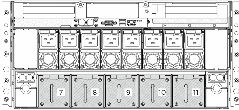
圖例 58. 後方風扇編號
