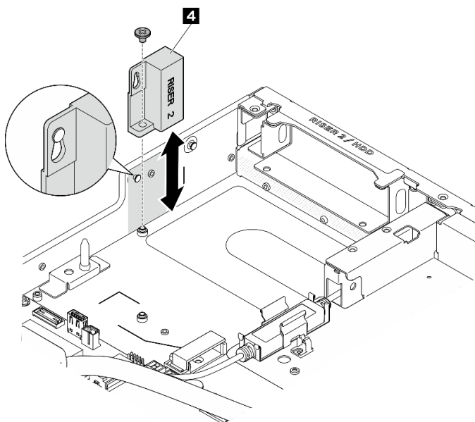
圖例 48. 將 DPU 空氣擋板安裝到機箱
