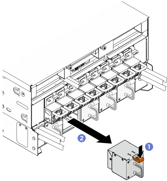
圖例 57. 卸下後方風扇
