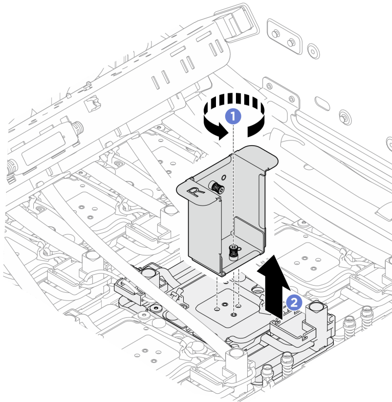
圖例 235. 卸下維修托架
