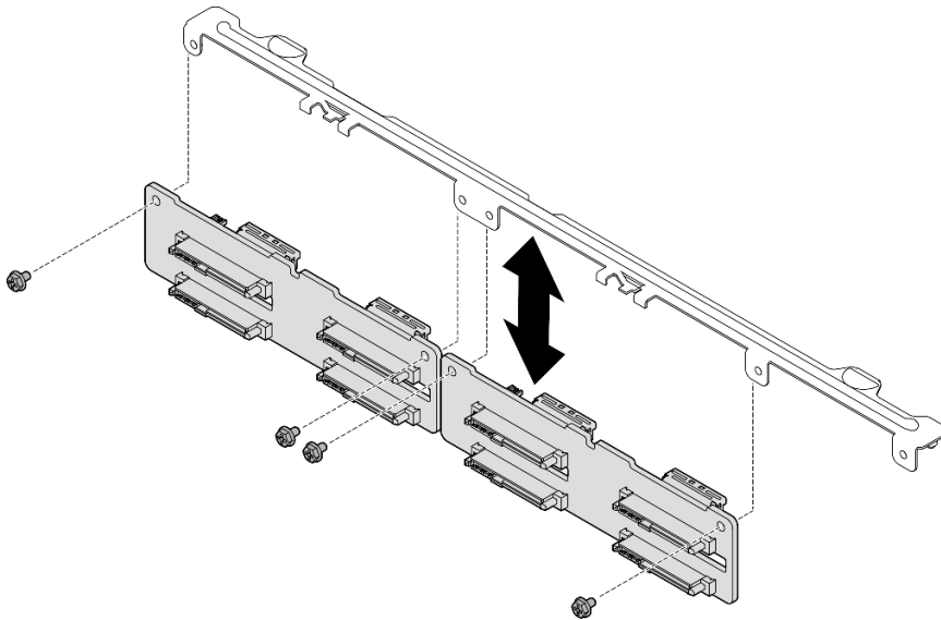
圖例 18. 卸下前方 2.5 吋硬碟背板
