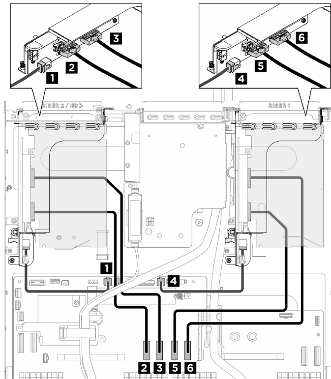
圖例 395. PCIe 擴充卡纜線佈線
