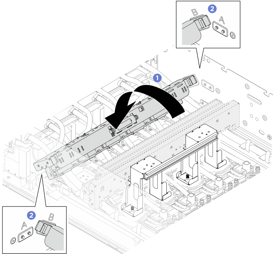
圖例 215. 重新放置後方 H100/H200 GPU 水冷板模組歧管
