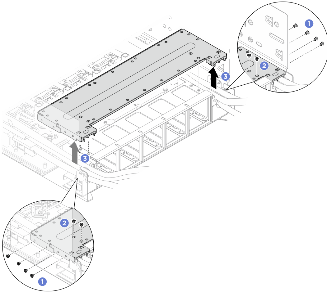
圖例 168. 卸下後方風扇機盒支撐托架
