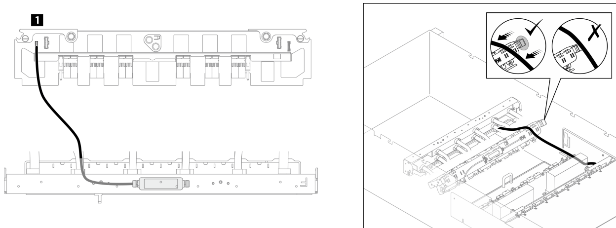
圖例 398. 前方 GPU 洩漏感應器模組纜線佈線
