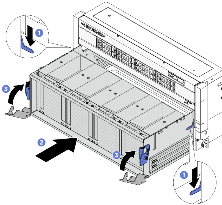
圖例 106. 安裝 PCIe 交換器滑動箱
