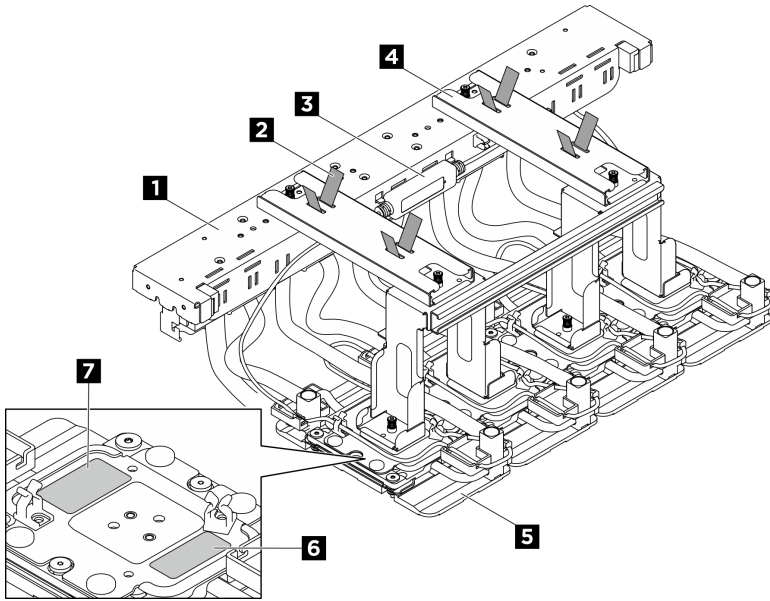
圖例 177. 後方 H100/H200 GPU 水冷板模組元件識別
