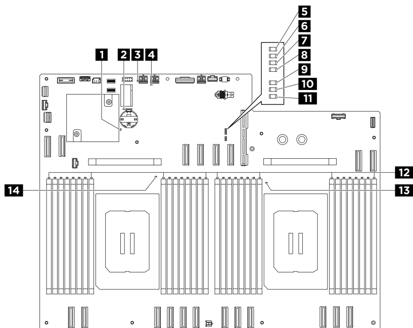
圖例 408. 主機板 LED
