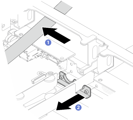
圖例 255. 拔開軟管
