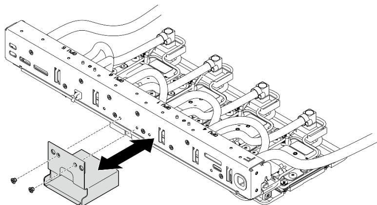
圖例 150. 安裝 GPU 纜線固定器
