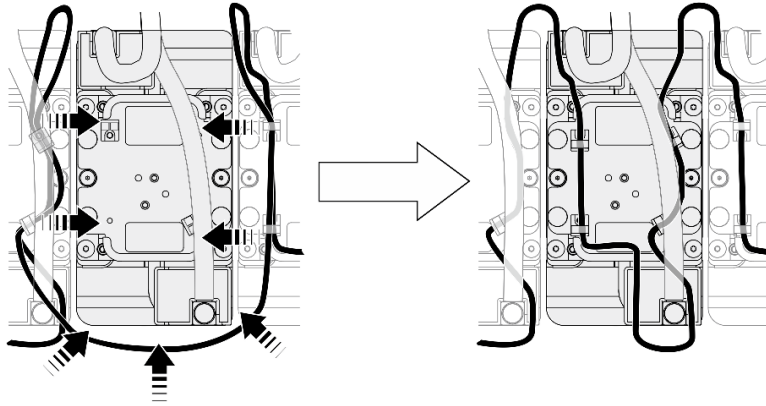
圖例 238. 安裝洩漏感應器模組纜線
