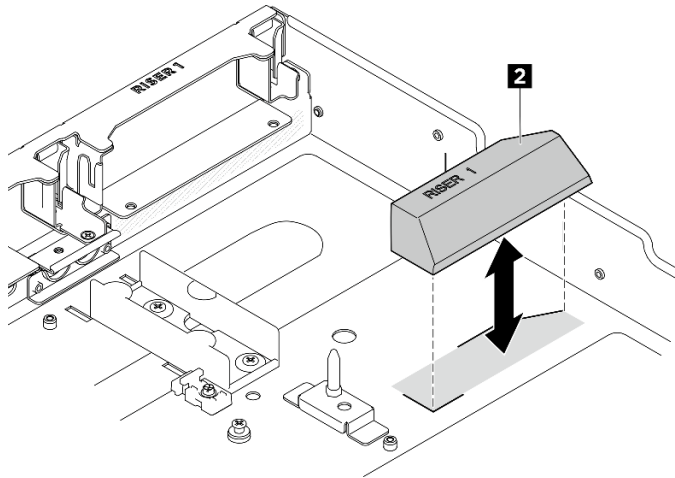
圖例 41. 將 DPU 空氣擋板安裝到機箱
