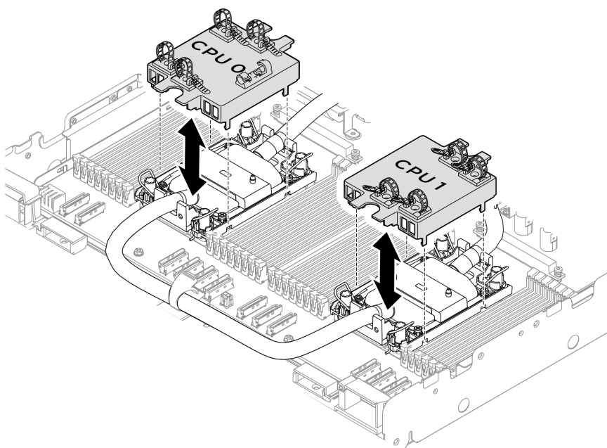
圖例 267. 安裝水冷板蓋
