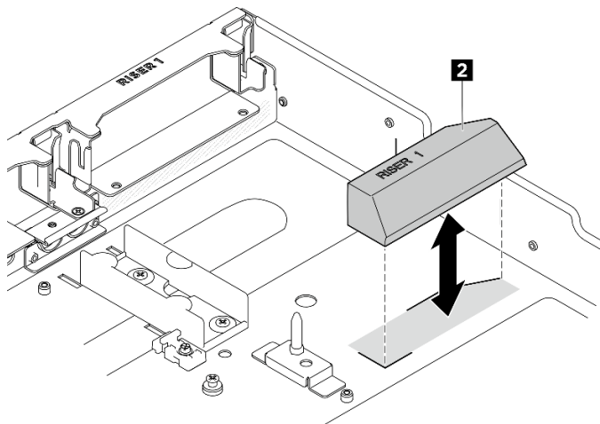
圖例 31. 從機箱卸下 DPU 空氣擋板
