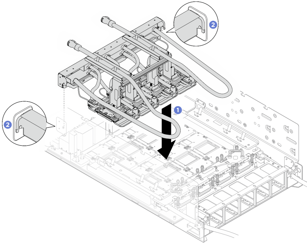
圖例 153. 安裝前方 H100/H200 GPU 水冷板模組
