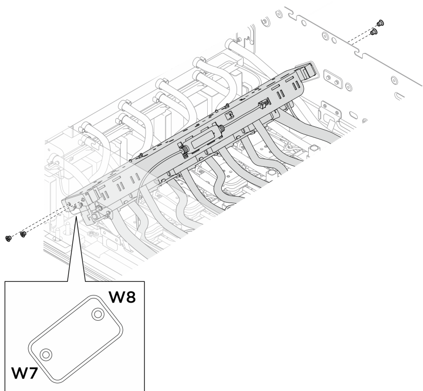
圖例 163. 安裝後方 H100/H200 GPU 水冷板模組歧管
