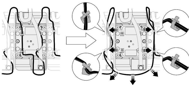
圖例 196. 移除洩漏感應器模組纜線
