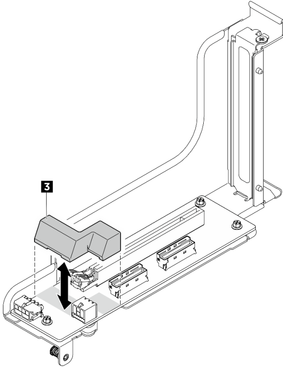
圖例 36. 從 PCIe 擴充卡卸下 DPU 空氣擋板
