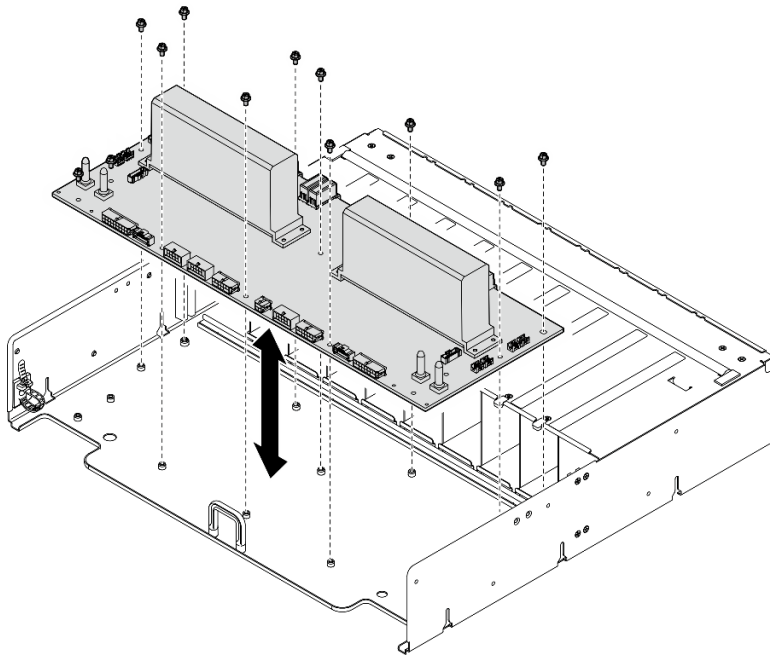
圖例 340. 安裝電源配送板
