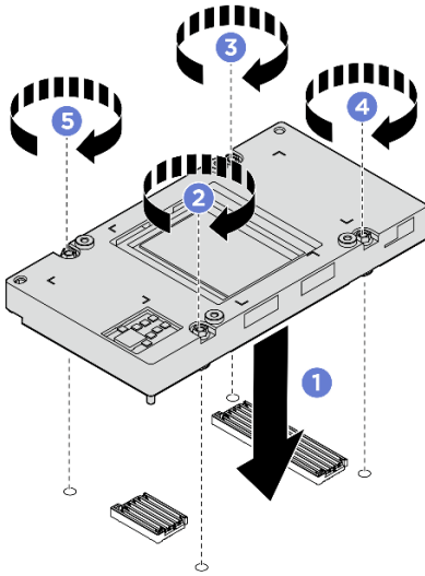
圖例 230. 安裝 GPU
