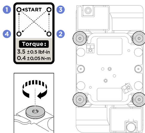
圖例 237. 安裝 GPU 水冷板
