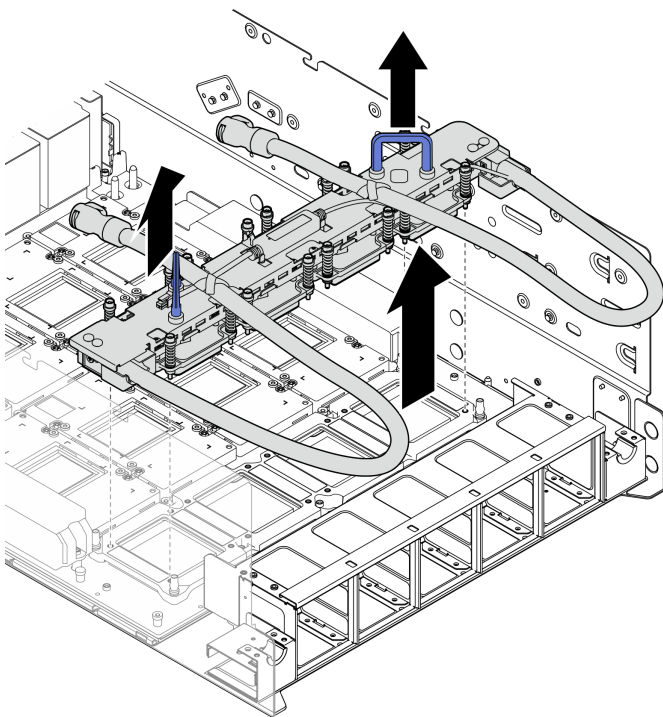
圖例 121. 卸下 NVSwitch 水冷板模組
