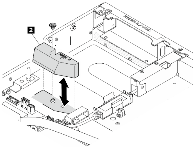
圖例 46. 將 DPU 空氣擋板安裝到機箱
