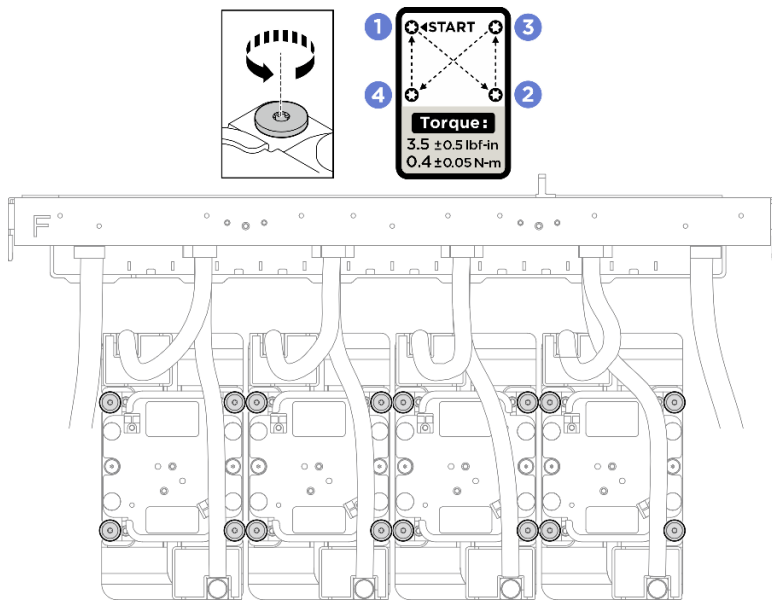
圖例 141. 卸下 GPU 水冷板
