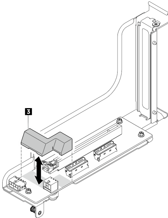
圖例 42. 將 DPU 空氣擋板安裝到 PCIe 擴充卡
