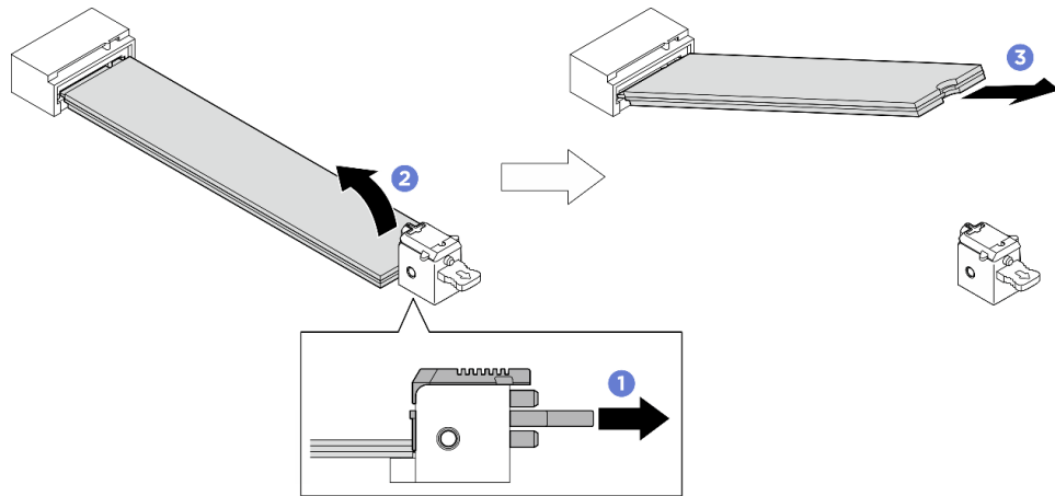
圖例 279. 卸下方 M.2 硬碟
