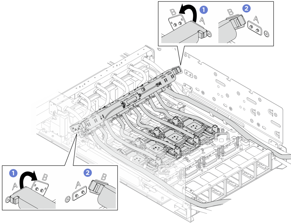
圖例 162. 重新安裝後方 H100/H200 GPU 水冷板模組歧管
