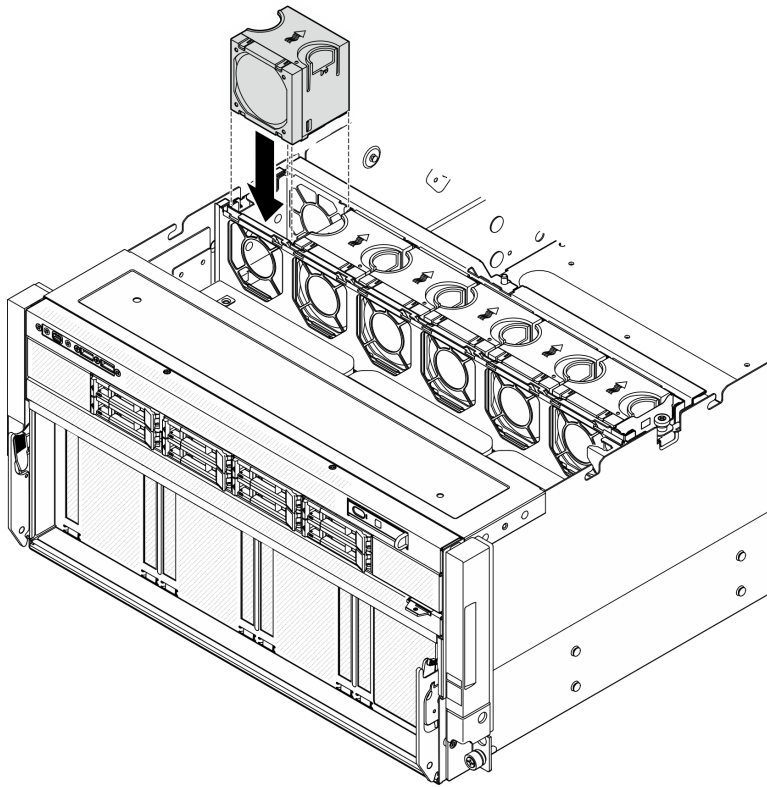
圖例 55. 前方風扇安裝
