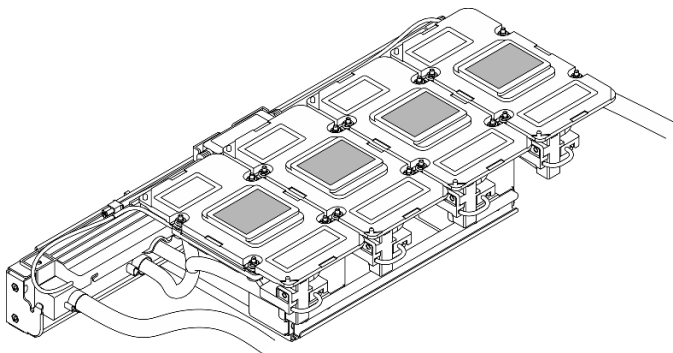
圖例 146. 擦掉水冷板上的 PCM 和油灰墊
