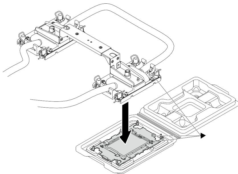
圖例 263. 組裝處理器與水冷板
