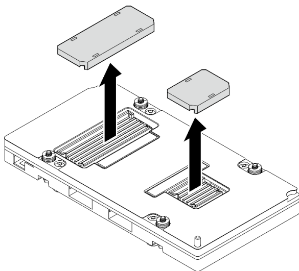
圖例 229. 移除接頭蓋
