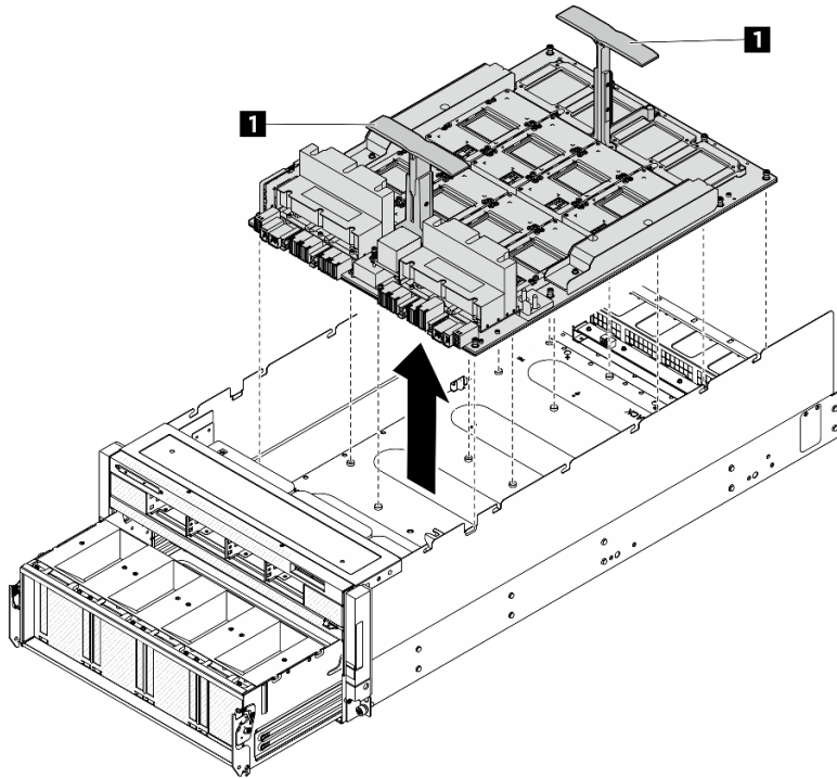
圖例 99. 卸下 GPU 複合體
