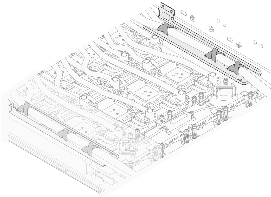
圖例 117. 將軟管和纜線從軟管束帶上鬆開
