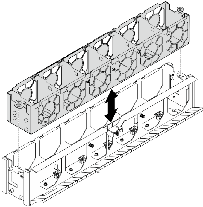
圖例 64. 安裝內部風扇機盒
