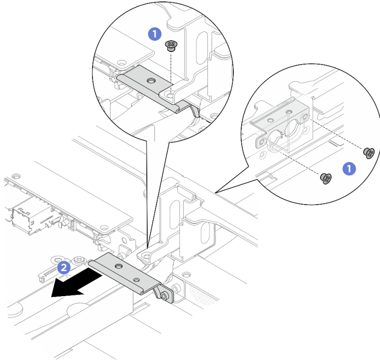
圖例 252. 卸下軟管蓋
