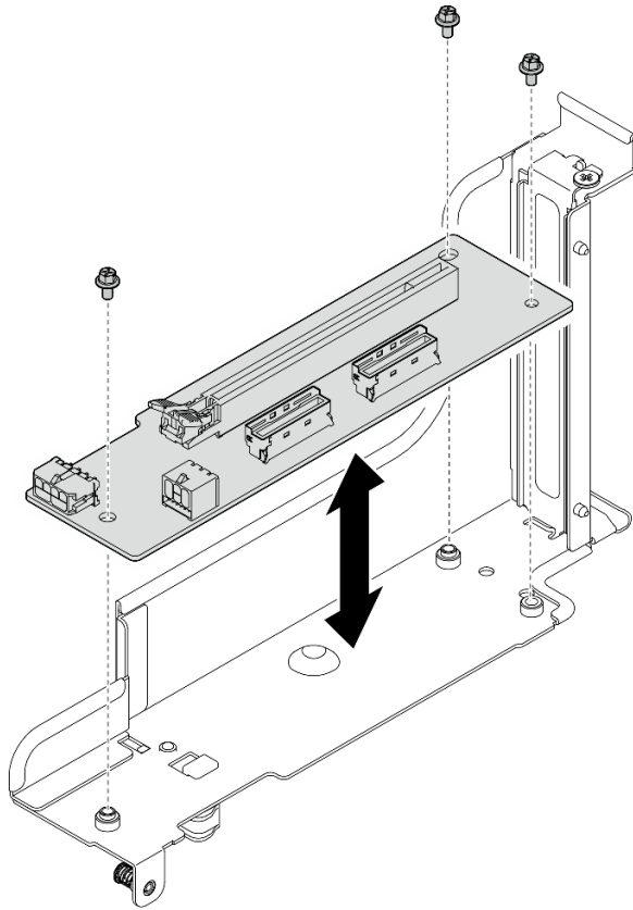
圖例 302. 卸下 PCIe 擴充卡
