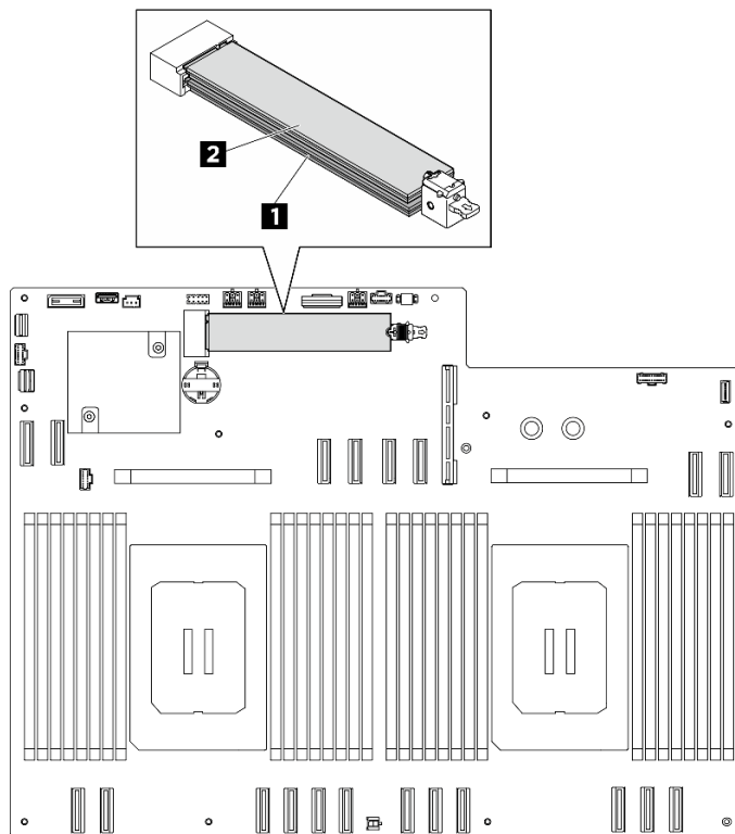
圖例 276. M.2 硬碟插槽
