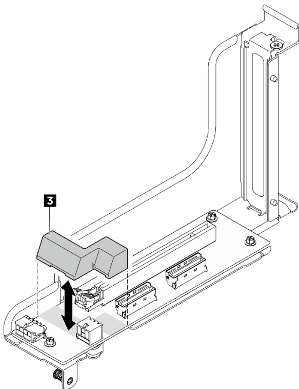
圖例 47. 將 DPU 空氣擋板安裝到 PCIe 擴充卡
