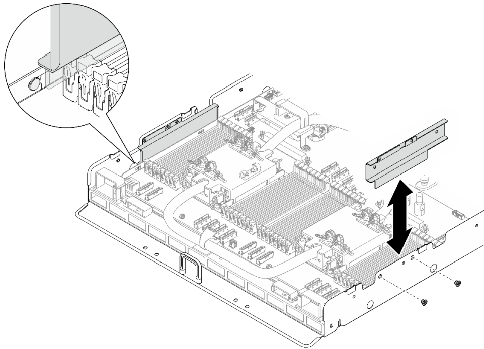
圖例 361. 卸下纜線導件
