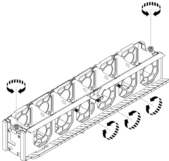
圖例 60. 分開內部風扇機盒
