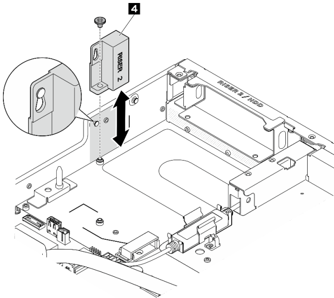
圖例 37. 從機箱卸下 DPU 空氣擋板
