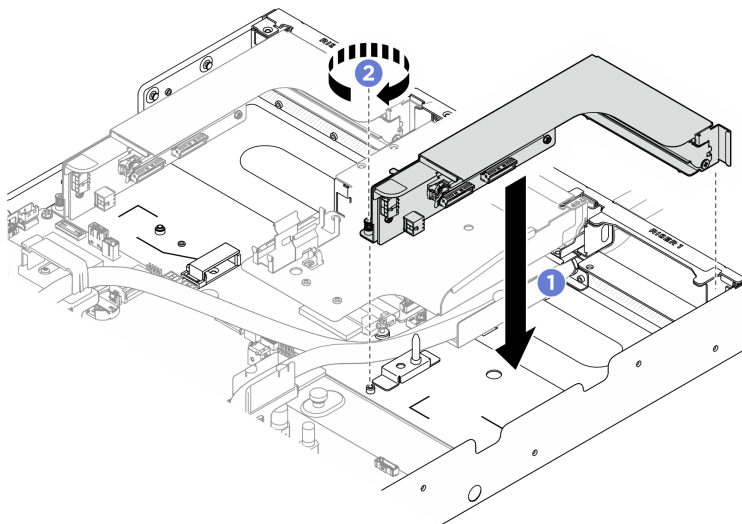
圖例 304. 將 PCIe 擴充卡組件安裝在插槽 1 中
