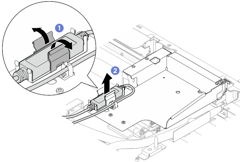
圖例 250. 鬆開洩漏感應器模組
