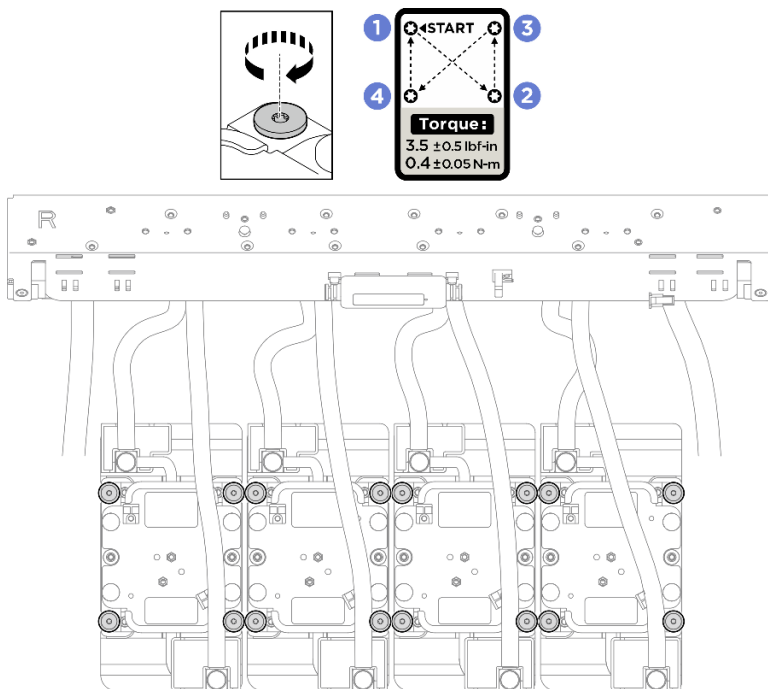
圖例 184. 安裝 GPU 水冷板
