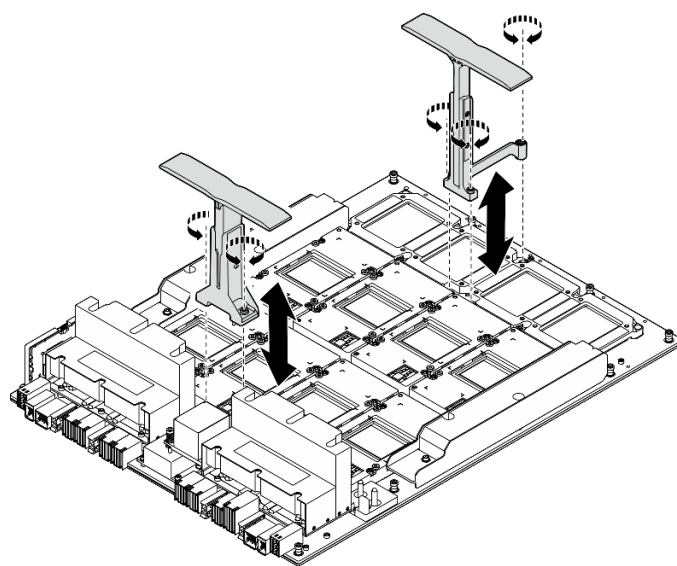
圖例 103. 卸下把手
