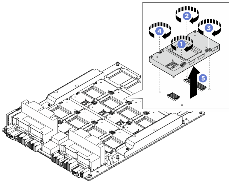
圖例 84. 卸下 GPU
