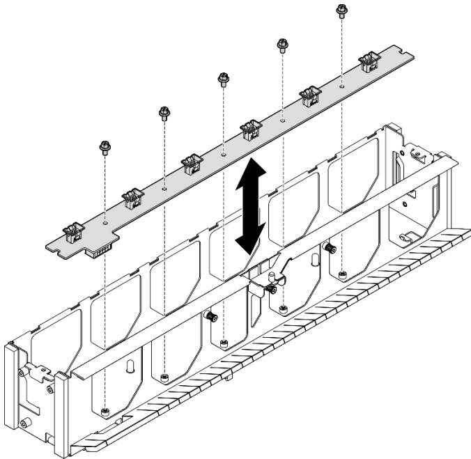
圖例 62. 卸下前方風扇控制板
