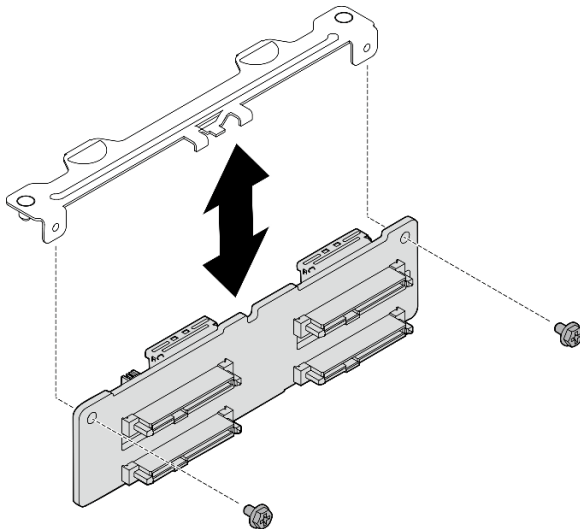
圖例 353. 安裝後方 2.5 吋硬碟背板
