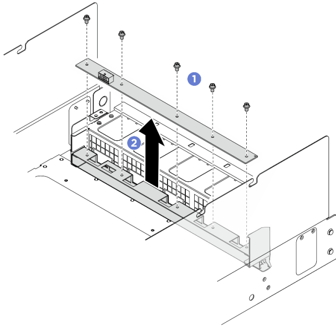
圖例 67. 卸下後方風扇控制板
