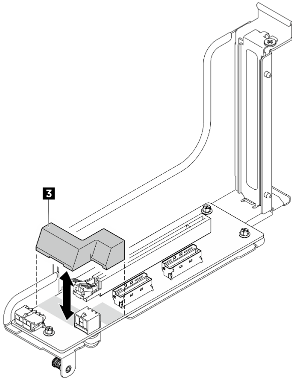
圖例 32. 從 PCIe 擴充卡卸下 DPU 空氣擋板
