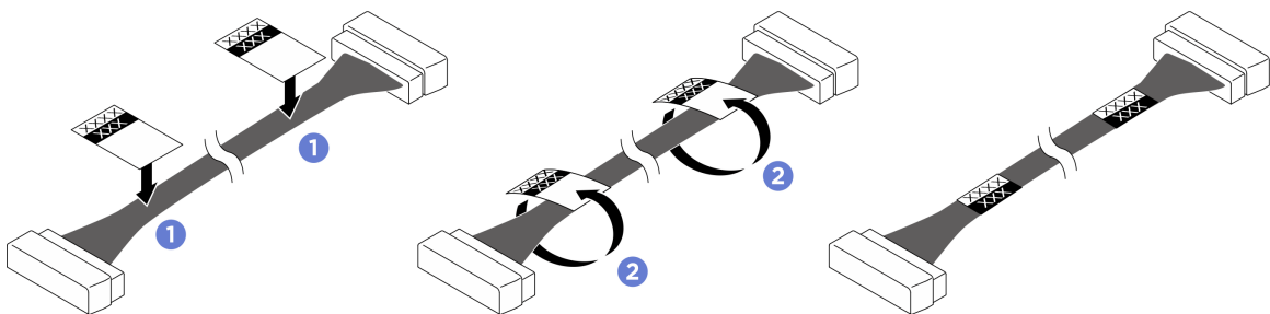
圖例 317. 黏貼標籤
