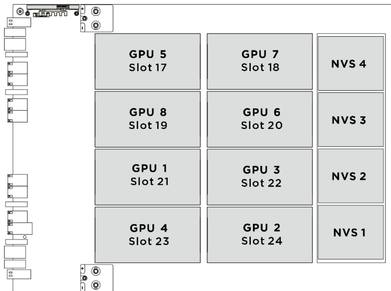
圖例 176. GPU 編號
