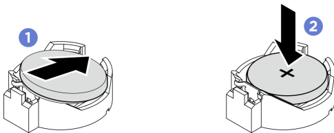
圖例 28. CMOS 電池安裝
