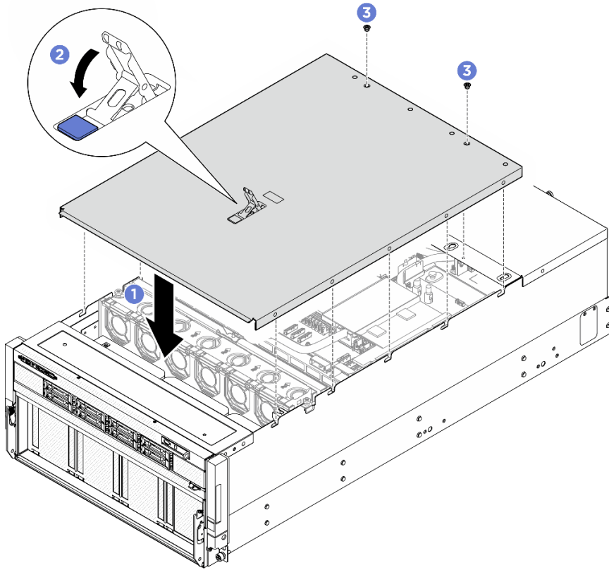
圖例 5. 安裝前方上蓋
