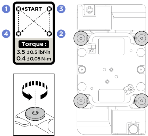
圖例 197. 卸下 GPU 水冷板
