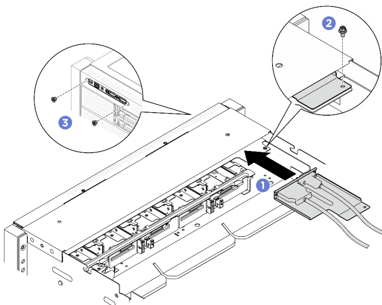
圖例 74. 安裝正面 I/O 模組
