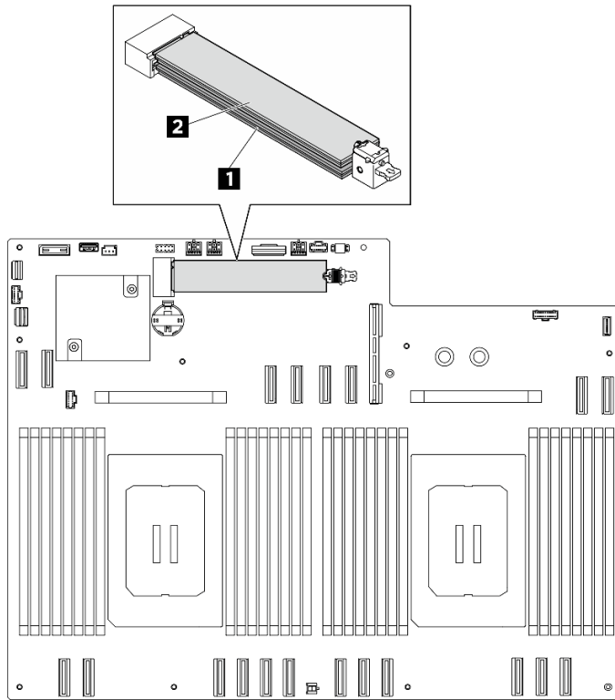
圖例 280. M.2 硬碟插槽
