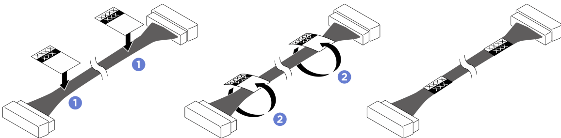
圖例 355. 黏貼標籤
