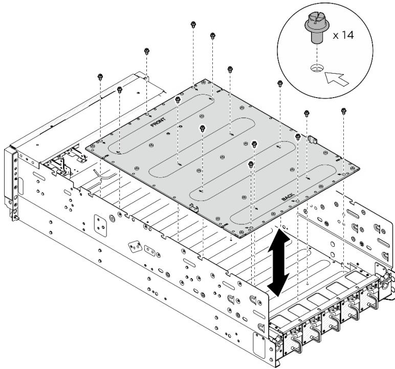
圖例 108. 卸下 GPU 複合體配接器板
