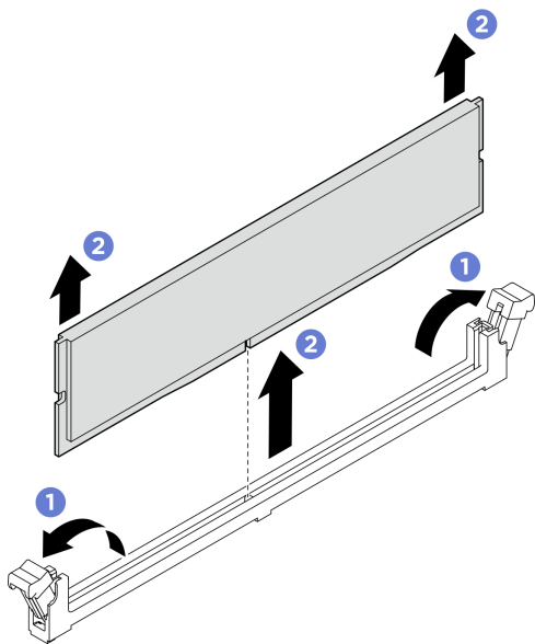
圖例 284. 卸下記憶體模組
