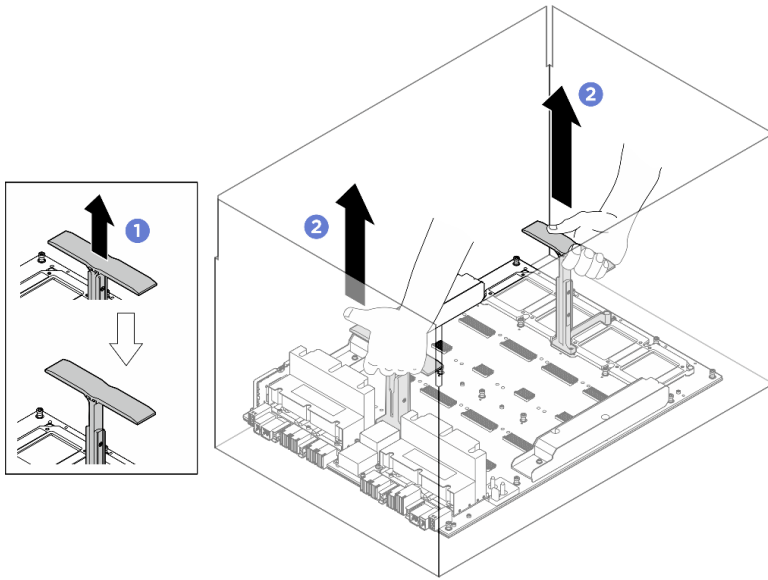
圖例 86. 從包裝盒中取出 GPU 基板
