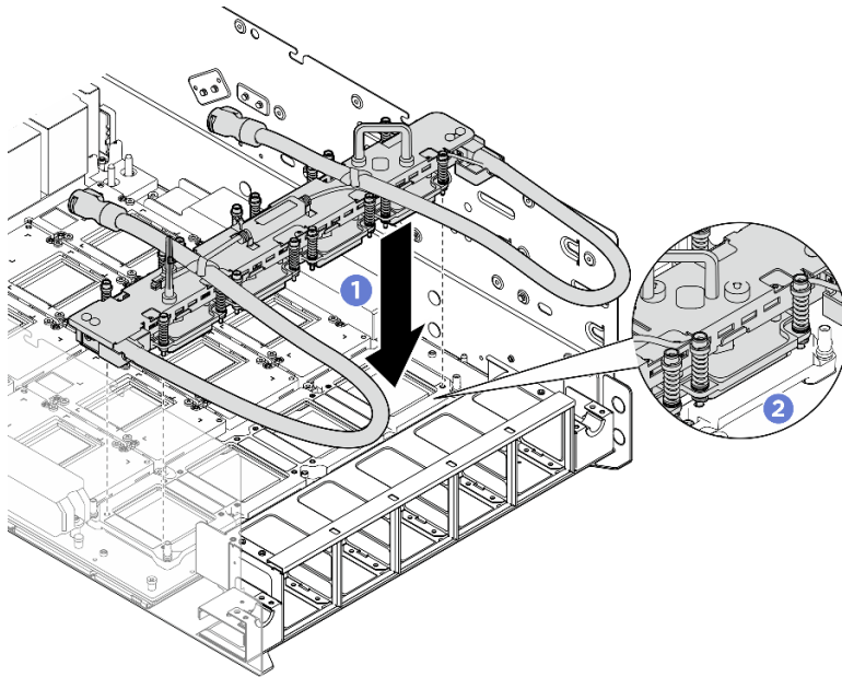
圖例 126. 安裝 NVSwitch 水冷板模組
