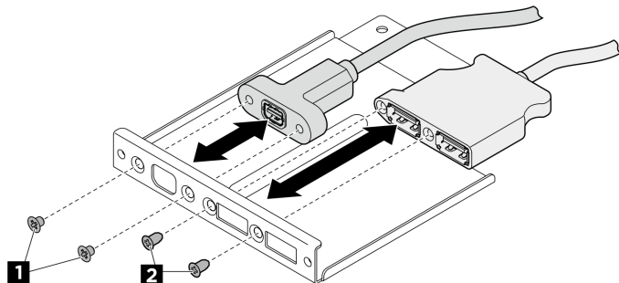
圖例 73. 安裝正面 I/O 模組纜線
