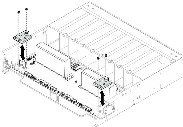
圖例 327. 安裝纜線固定器
