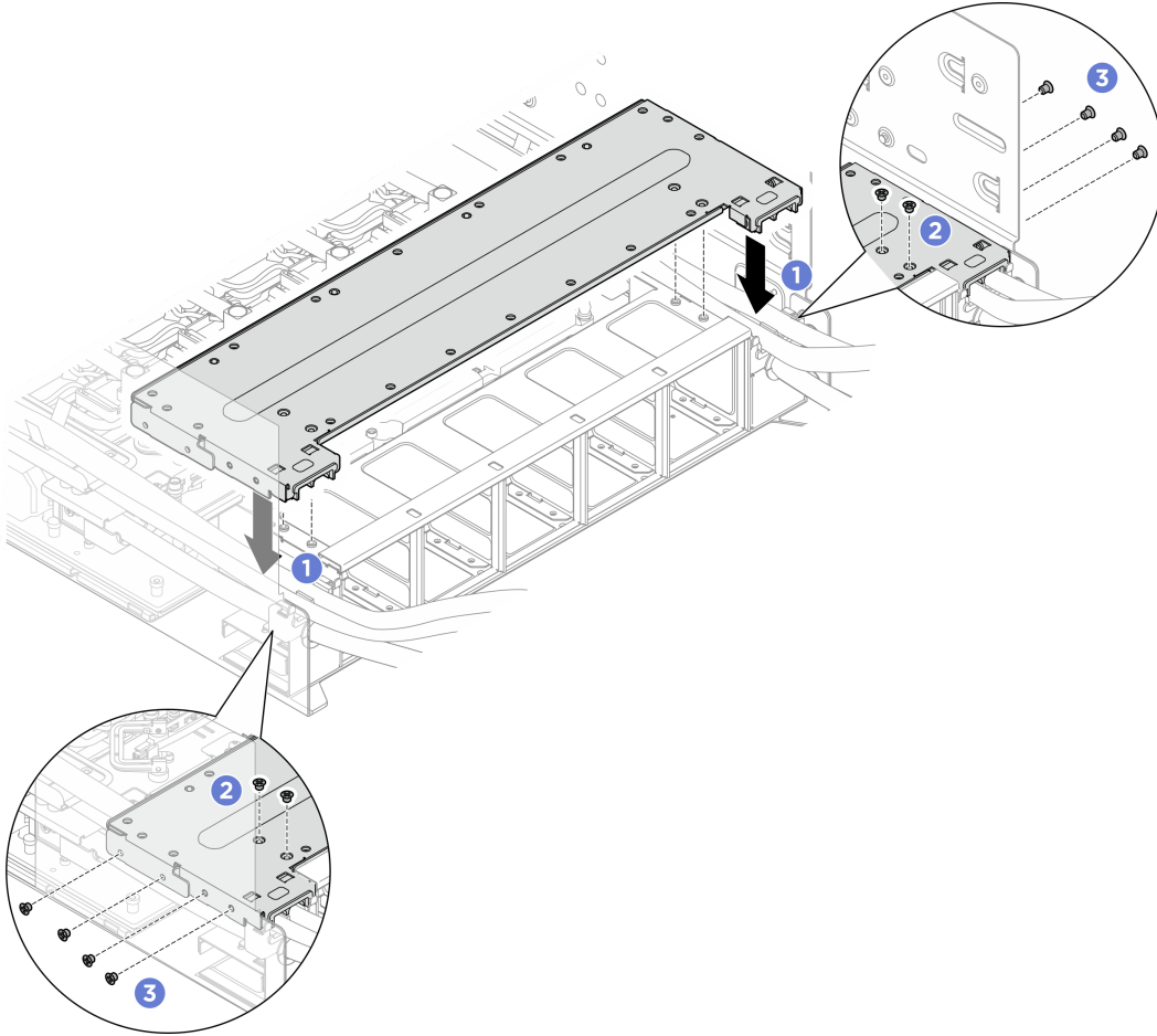
圖例 190. 安裝後方風扇機盒支撐托架
