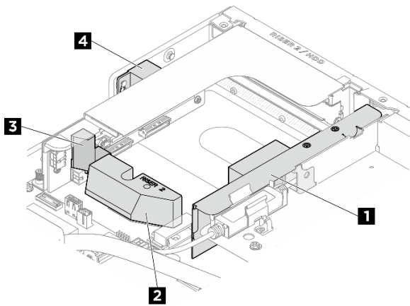
圖例 33. DPU 空氣擋板在擴充卡 2 插槽中的位置
