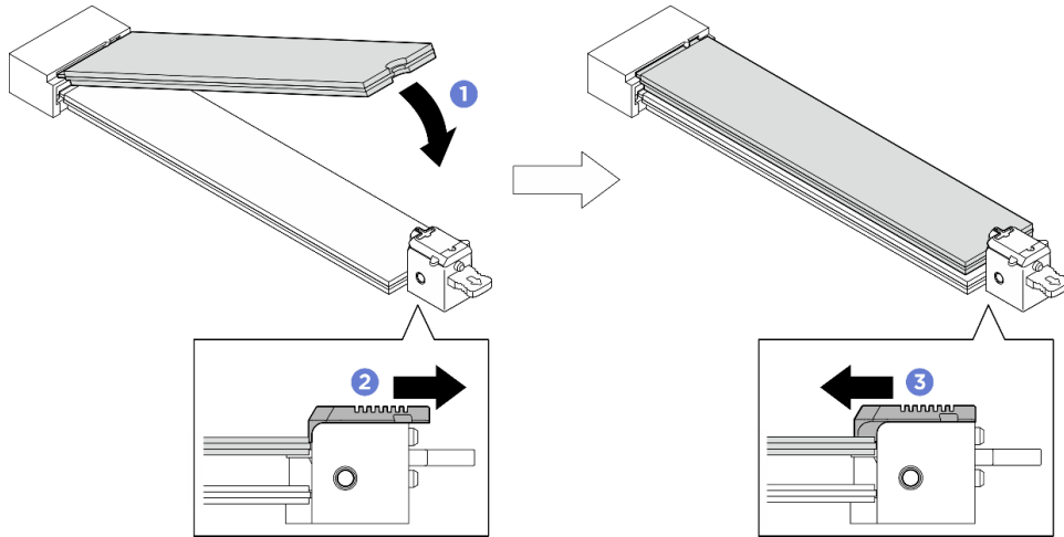
圖例 282. 安裝上方 M.2 硬碟
