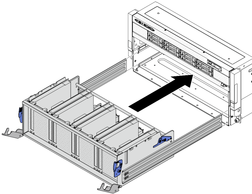
圖例 316. 將 PCIe 交換器滑動箱安裝到停止位置
