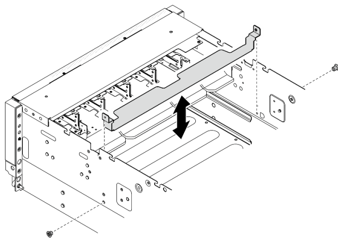
圖例 126. 安裝 GPU 接頭保護托架
