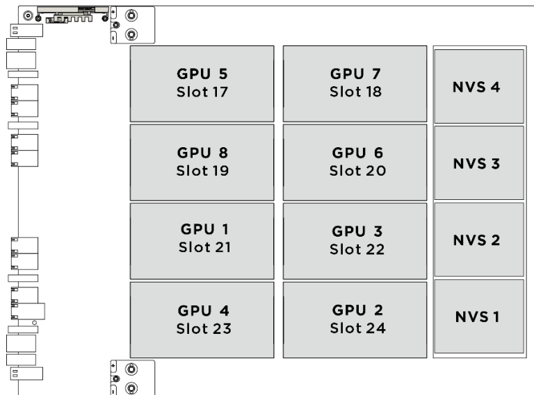
圖例 145. GPU 編號
