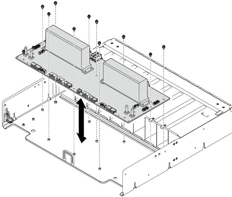
圖例 361. 安裝電源配送板
