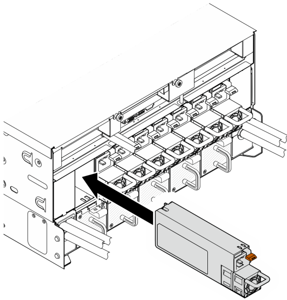
圖例 354. 安裝電源供應器
