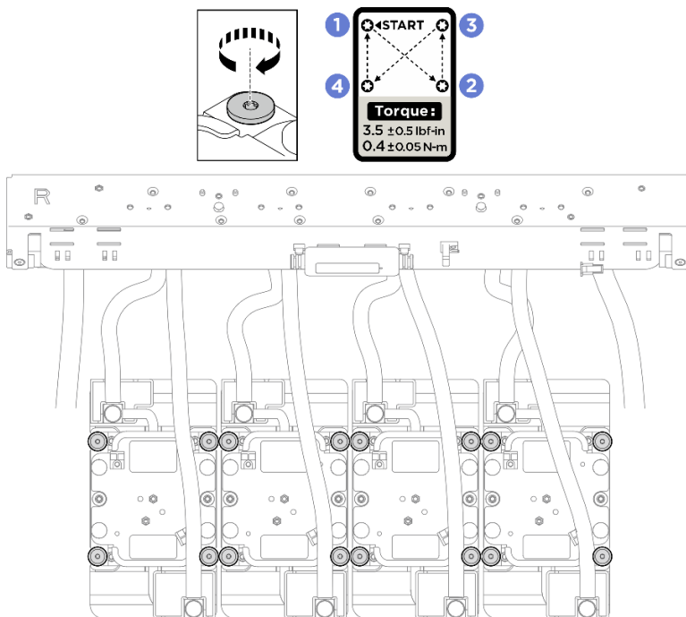
圖例 205. 安裝 GPU 水冷板
