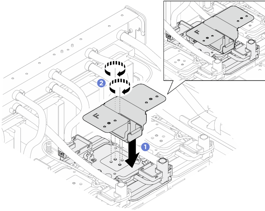
圖例 219. 將維修托架安裝到 GPU 水冷板上
