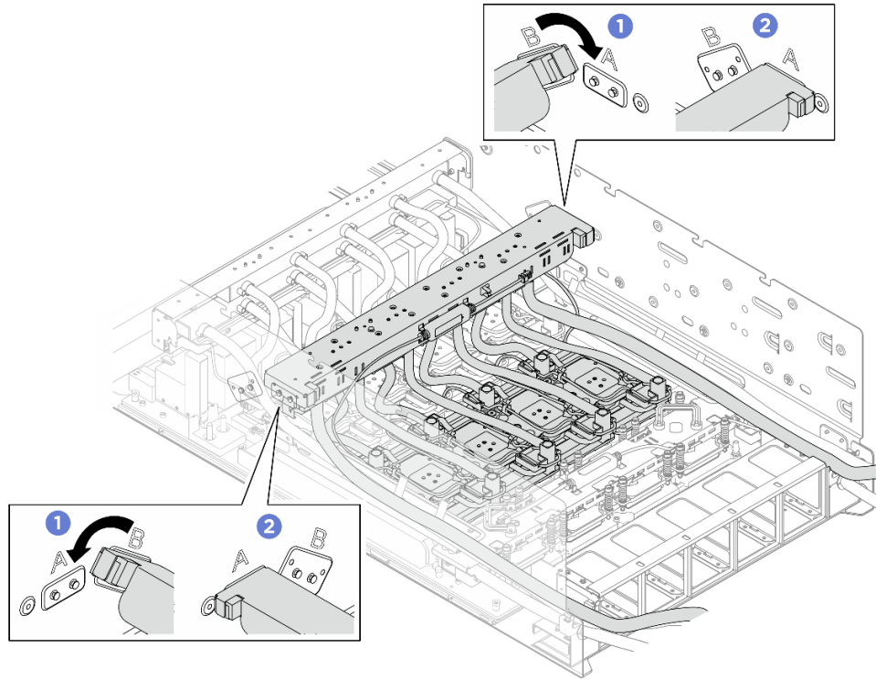
圖例 161. 重新放置後方 H100/H200 GPU 水冷板模組歧管
