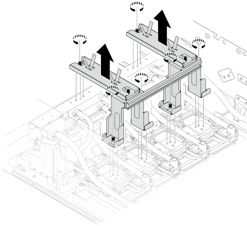
圖例 176. 卸下出貨托架
