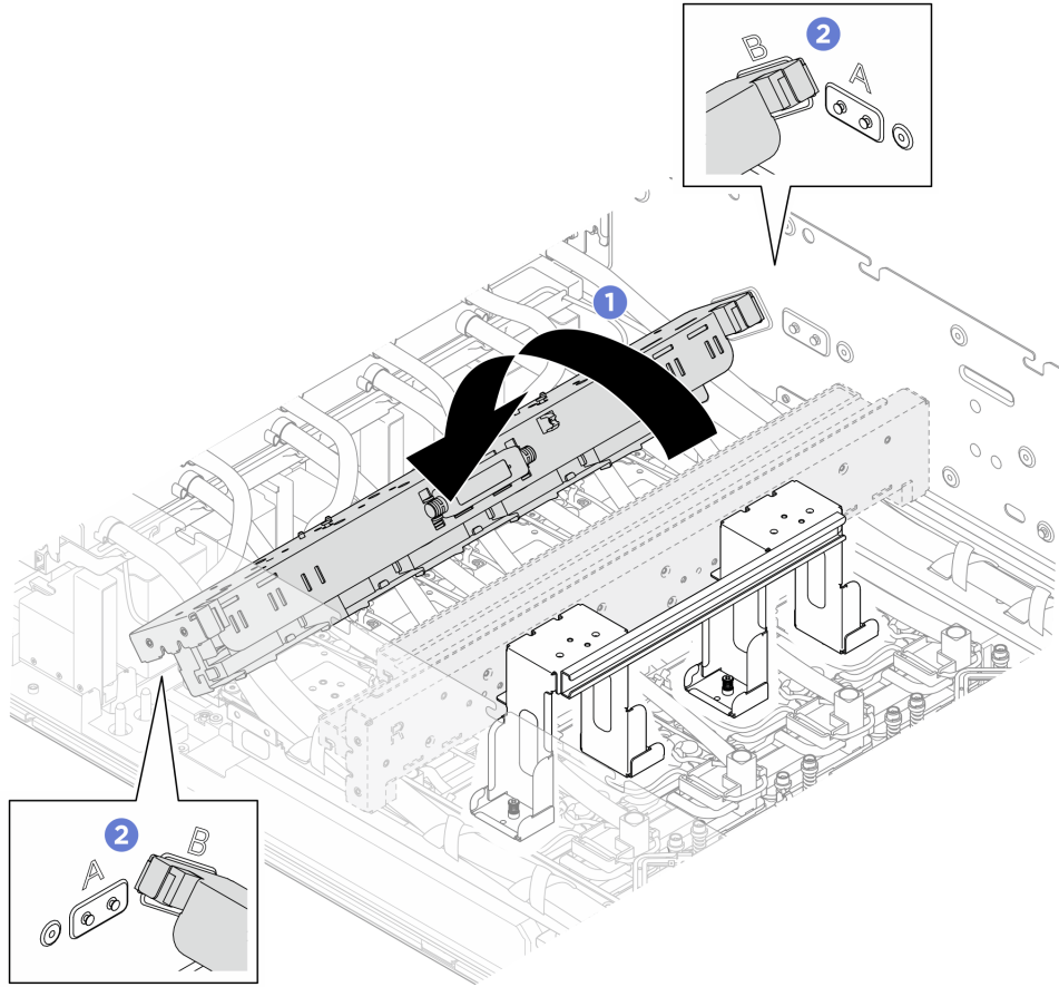
圖例 236. 重新放置後方 H100/H200 GPU 水冷板模組歧管
