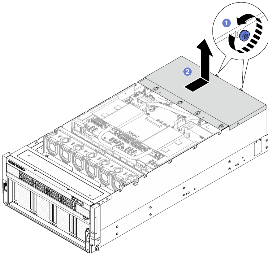
圖例 27. 卸下後方上蓋
