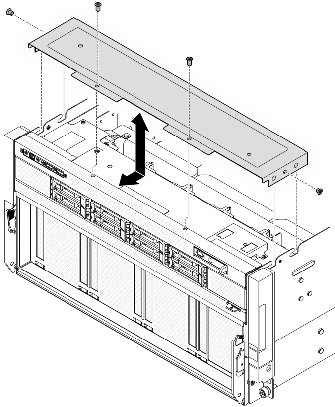
圖例 265. 卸下 I/O 蓋板
