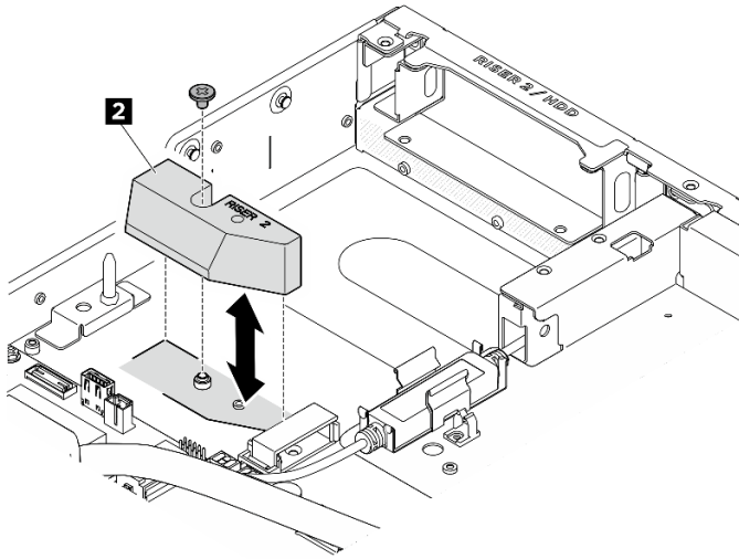
圖例 56. 從機箱卸下 DPU 空氣擋板
