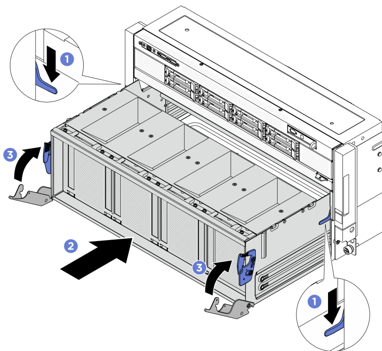
圖例 114. 安裝 PCIe 交換器滑動箱
