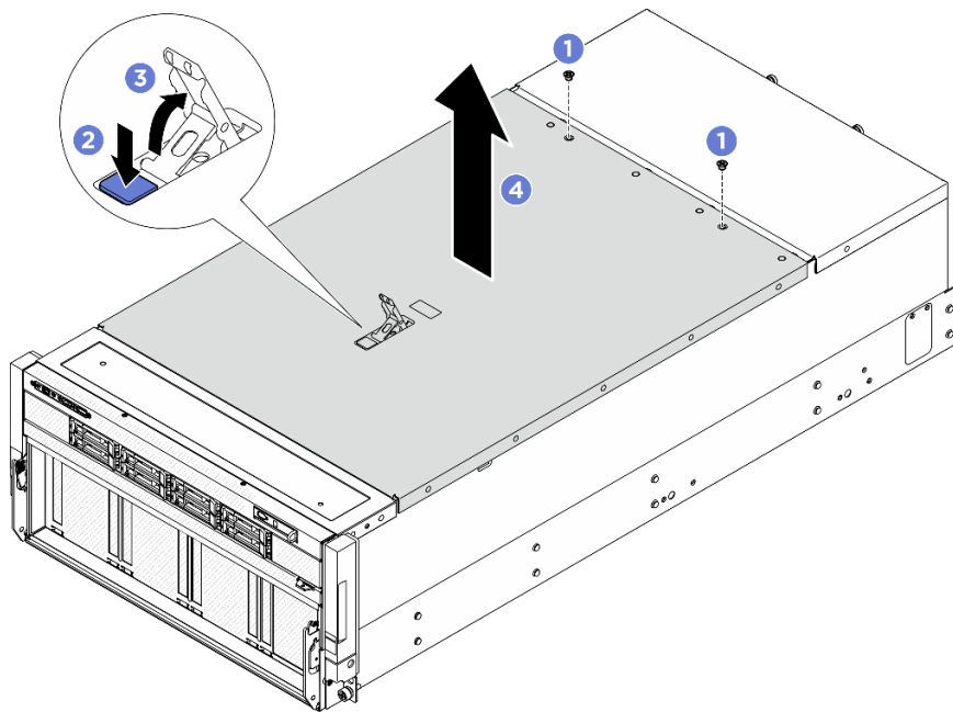
圖例 25. 卸下前方上蓋
