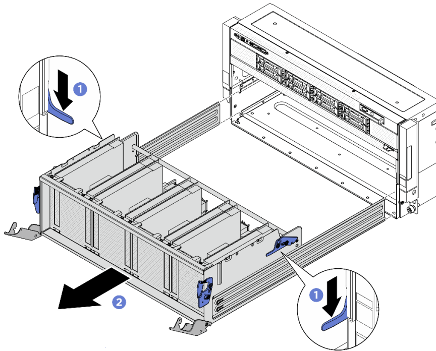
圖例 336. 卸下 PCIe 交換器滑動箱
