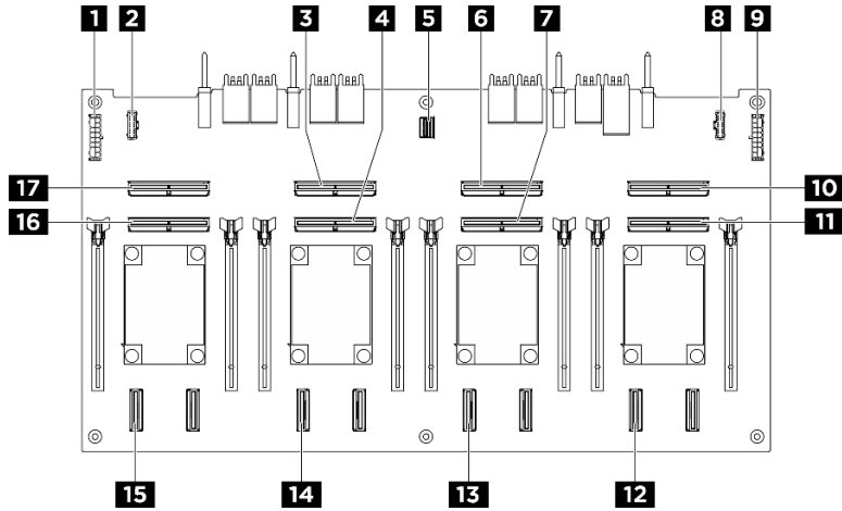
圖例 396. PCIe 交換器板接頭
