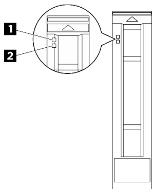
圖例 429. 硬碟 LED
