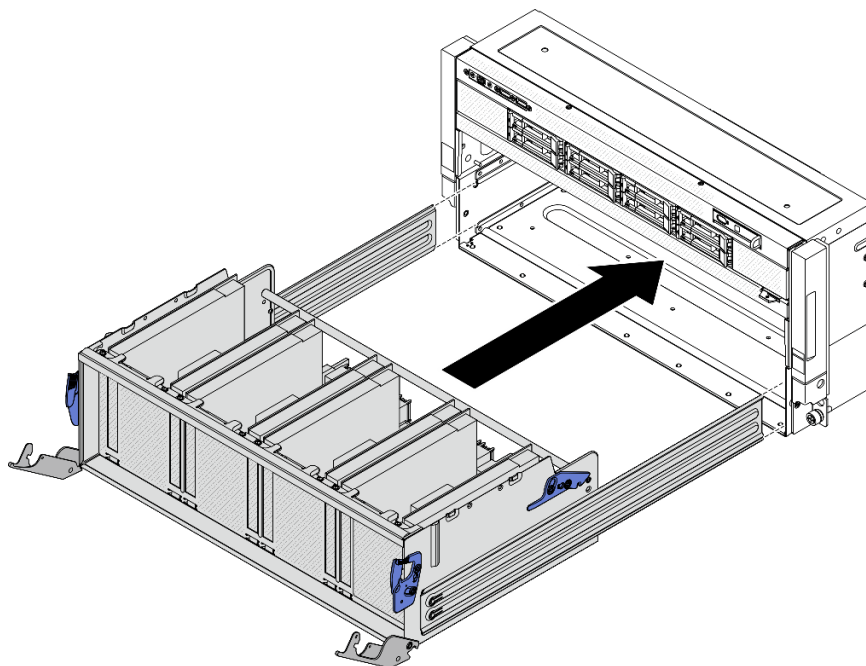
圖例 337. 將 PCIe 交換器滑動箱安裝到停止位置
