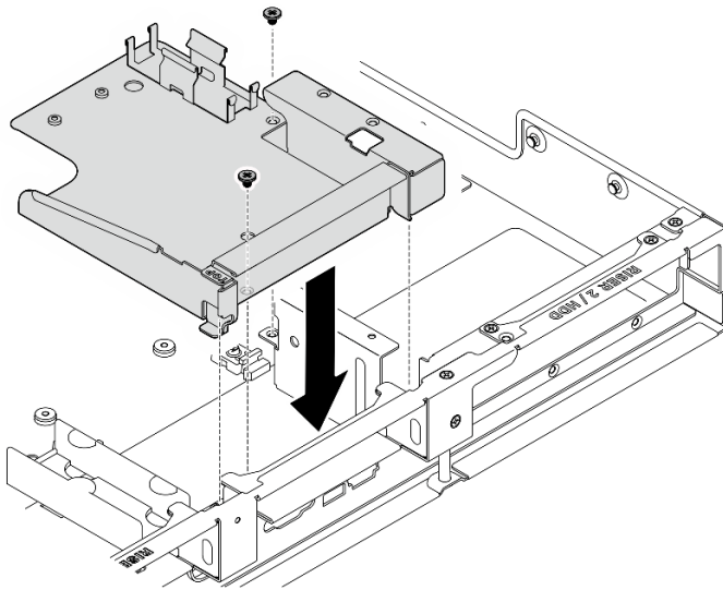
圖例 378. 安裝洩漏感應器模組托架
