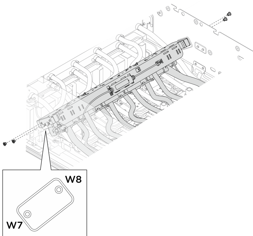
圖例 160. 卸下後方 H100/H200 GPU 水冷板模組歧管
