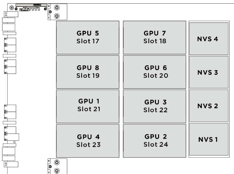
圖例 106. GPU 編號
