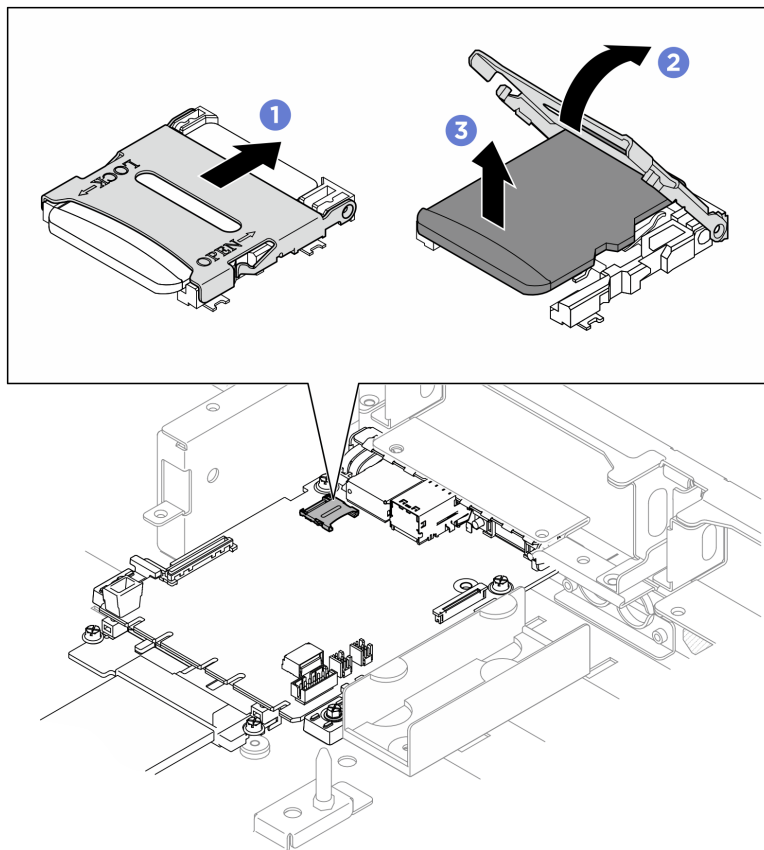
圖例 308. 卸下 MicroSD 卡
