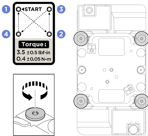
圖例 242. 卸下 GPU 水冷板
