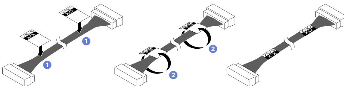
圖例 338. 黏貼標籤
