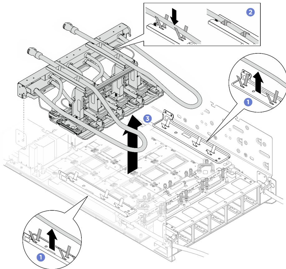
圖例 165. 卸下前方 H100/H200 GPU 水冷板模組
