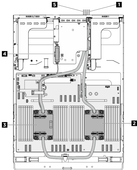
圖例 7. CPU 複合體水迴路俯視圖
