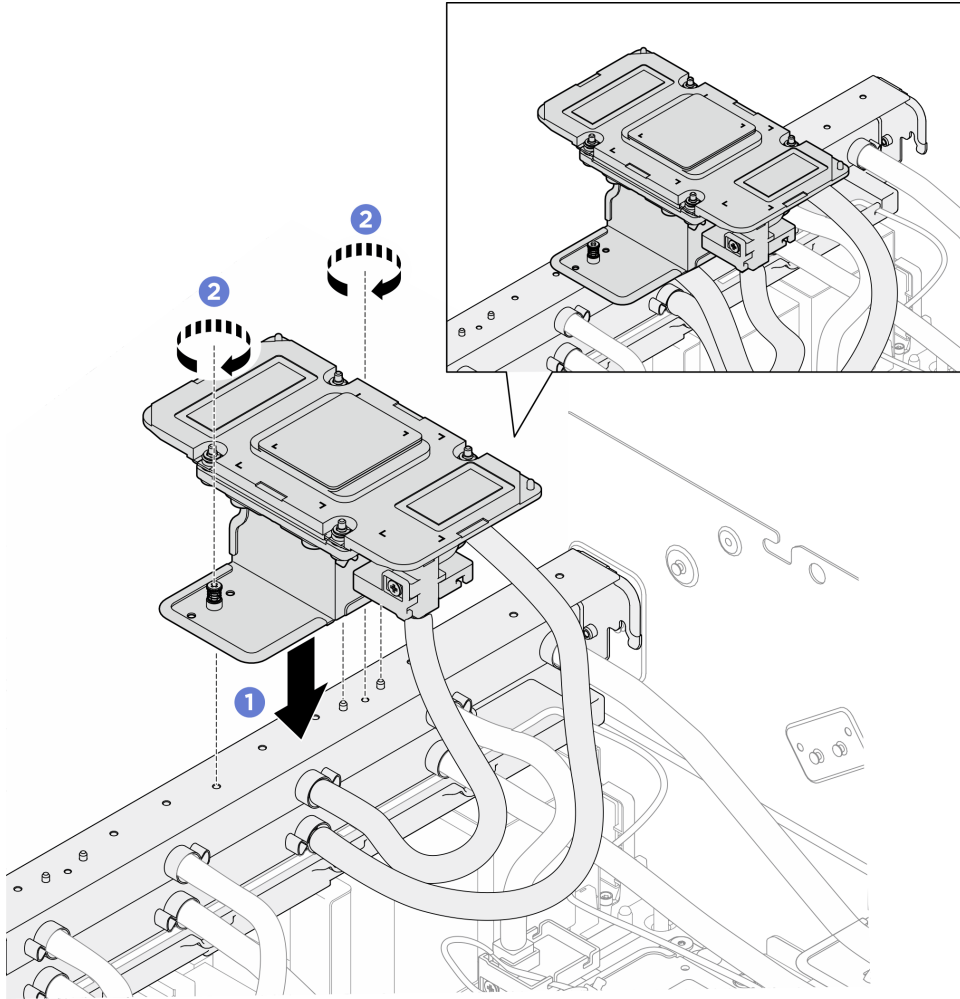
圖例 220. 安裝維修托架和 GPU 水冷板組件
