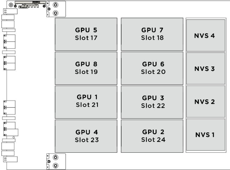
圖例 212. GPU 編號
