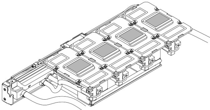
圖例 167. 擦掉水冷板上的 PCM 和油灰墊
