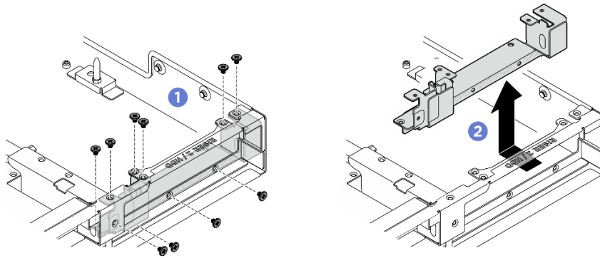
圖例 321. 卸下背面擴充卡支撐托架
