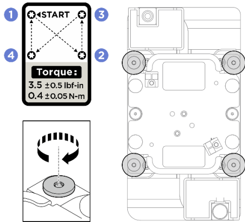
圖例 234. 安裝 GPU 水冷板
