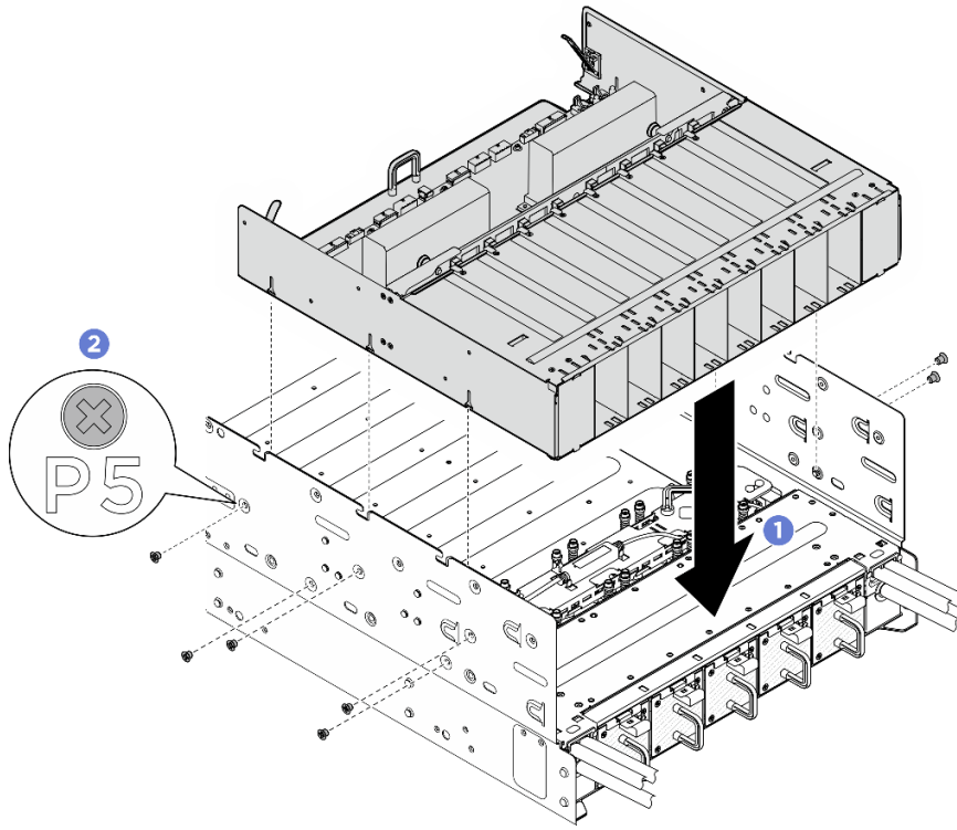
圖例 364. 安裝電源複合體
