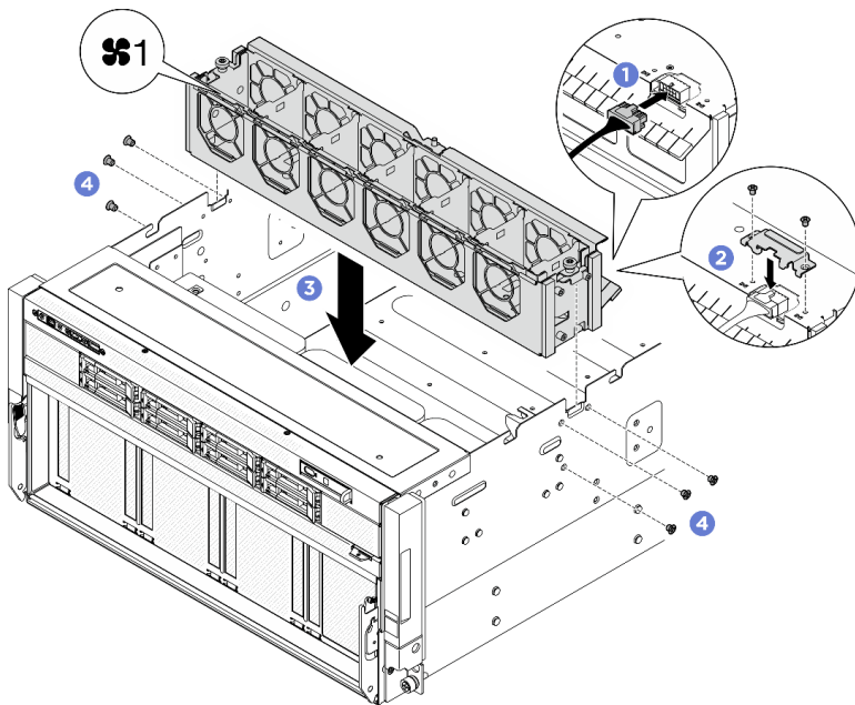
圖例 73. 安裝風扇機盒
