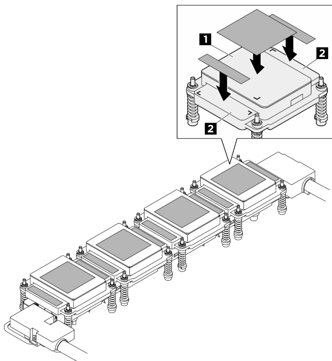
圖例 146. 貼附 PCM 和油灰墊
