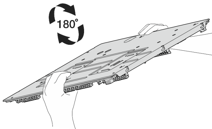
圖例 441. 將主機板組件轉至正面朝上
