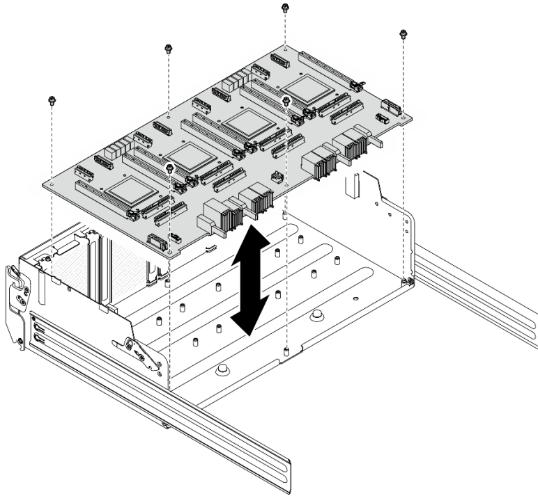
圖例 330. 卸下 PCIe 交換器板
