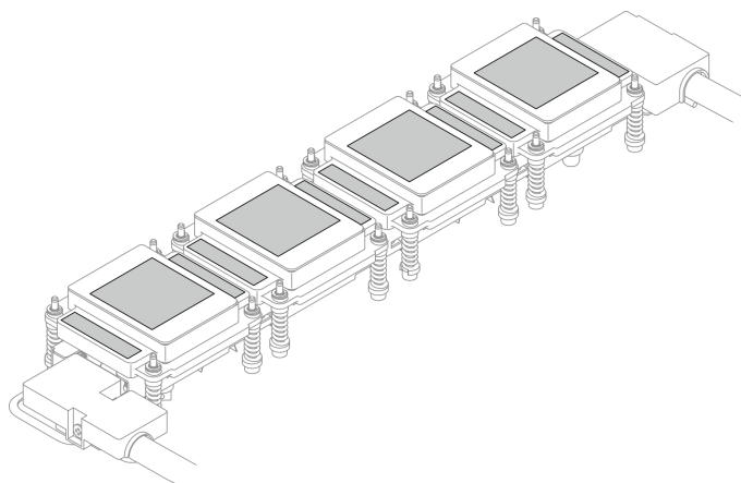
圖例 144. 擦掉水冷板上的 PCM 和油灰墊
