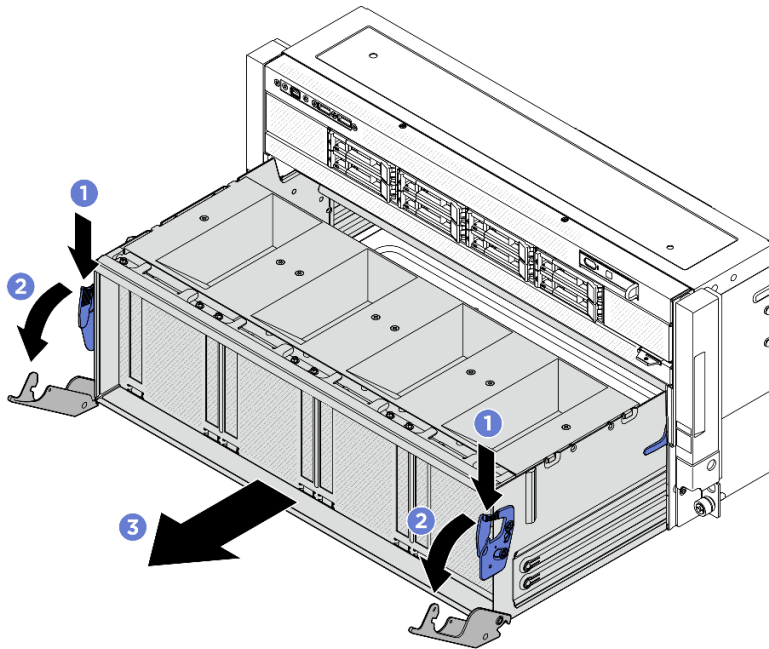
圖例 115. 將 PCIe 交換器滑動箱從停止位置卸下
