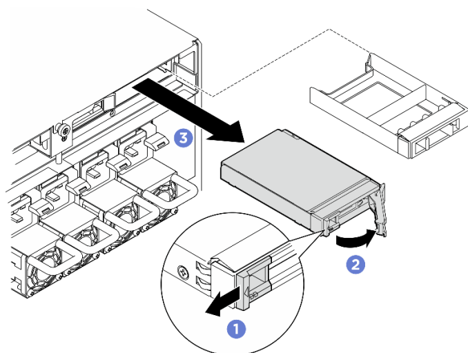
圖例 32. 卸下後方 2.5 吋熱抽換硬碟
