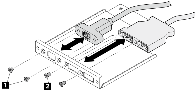
圖例 94. 安裝正面 I/O 模組纜線
