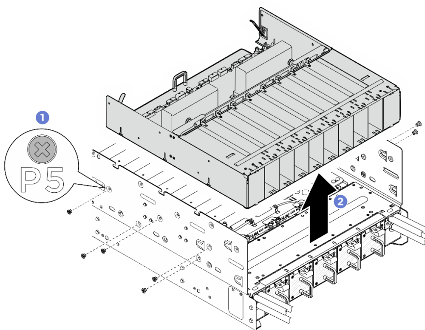
圖例 357. 卸下電源複合體
