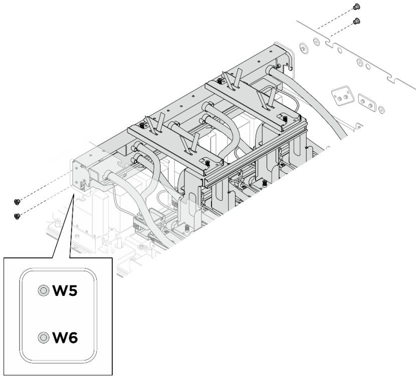
圖例 175. 安裝前方 H100/H200 GPU 水冷板模組歧管
