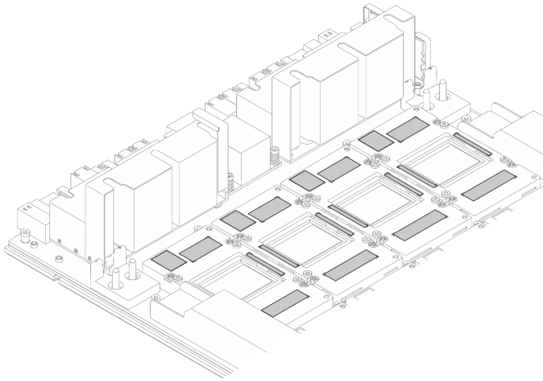
圖例 166. 清除 GPU 上的 PCM 和油灰墊
