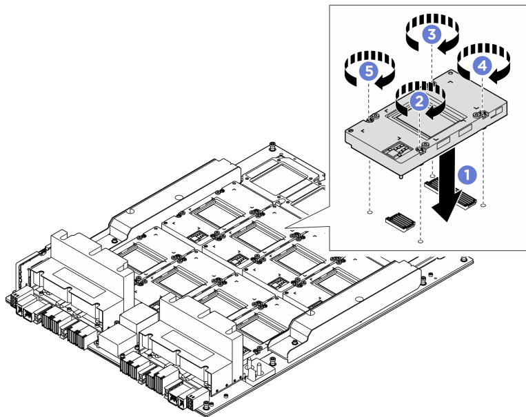
圖例 108. 安裝 GPU
