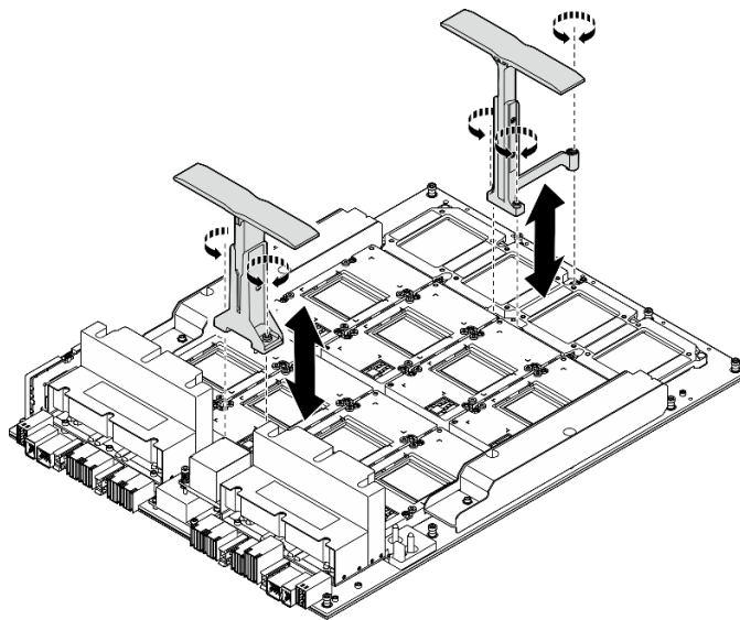
圖例 119. 安裝把手
