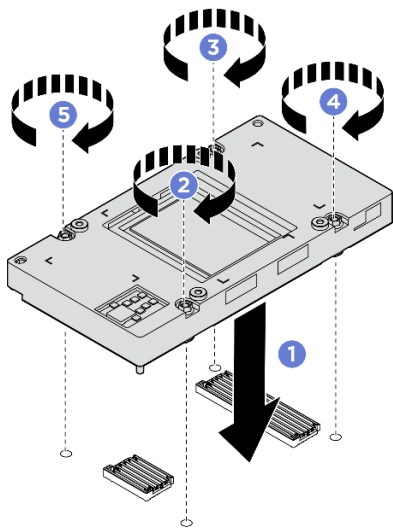
圖例 251. 安裝 GPU
