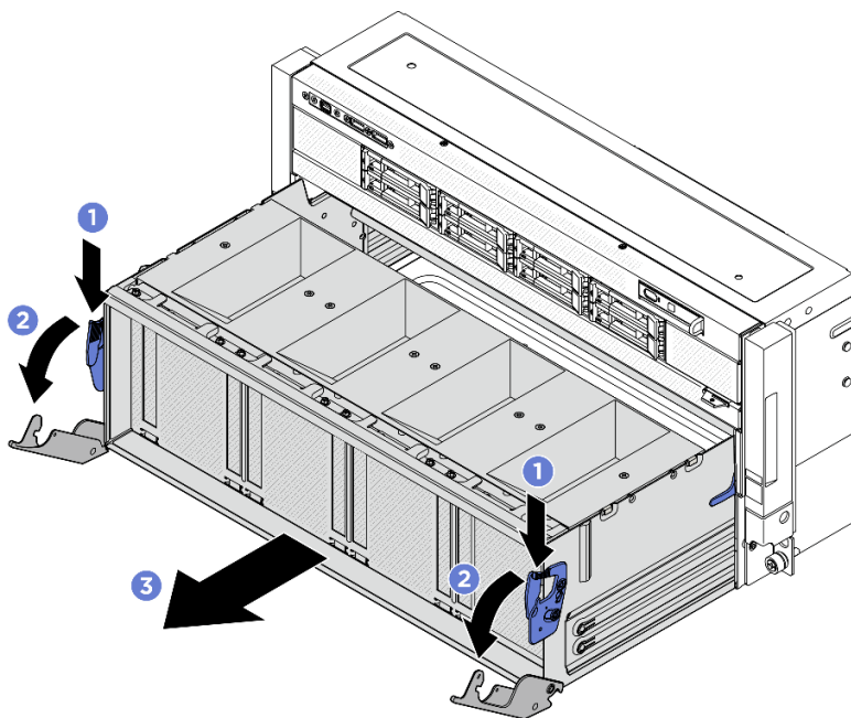
圖例 310. 將 PCIe 交換器滑動箱從停止位置卸下
