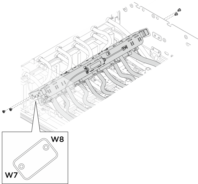
圖例 191. 卸下後方 H100/H200 GPU 水冷板模組歧管
