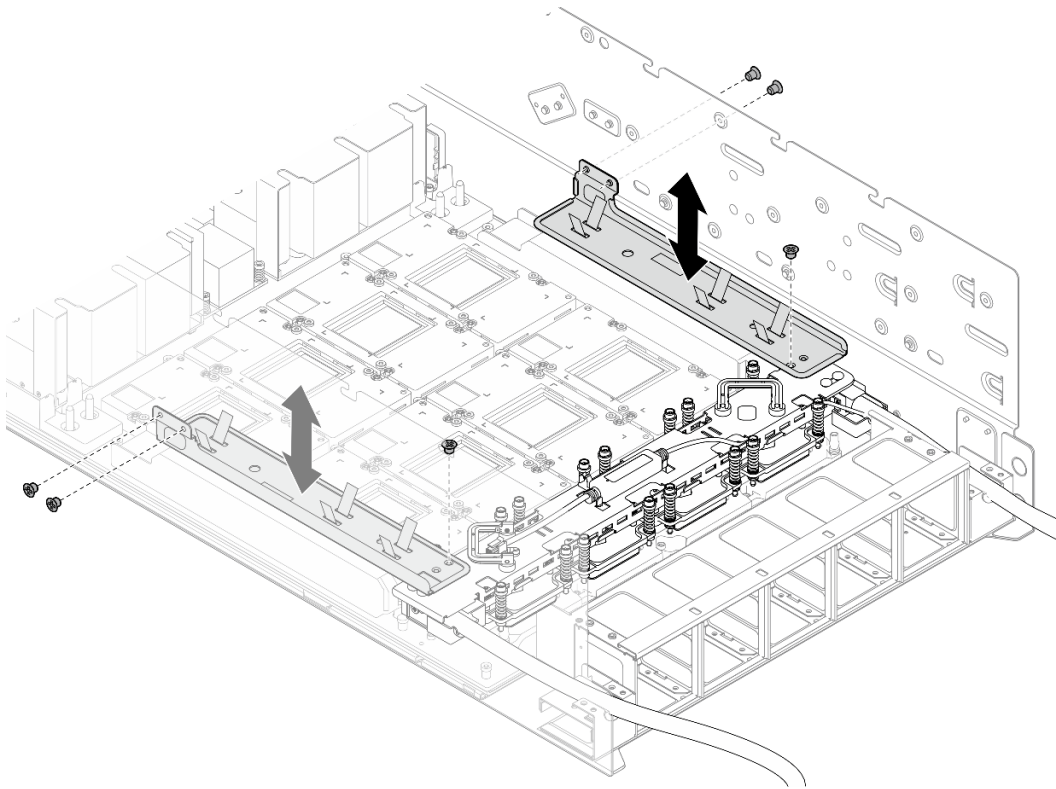
圖例 139. 卸下軟管導管
