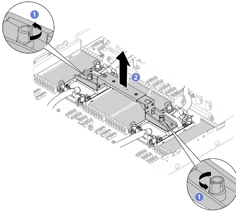
圖例 287. 卸下模組把手
