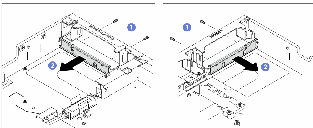
圖例 388. 卸下排氣區塊
