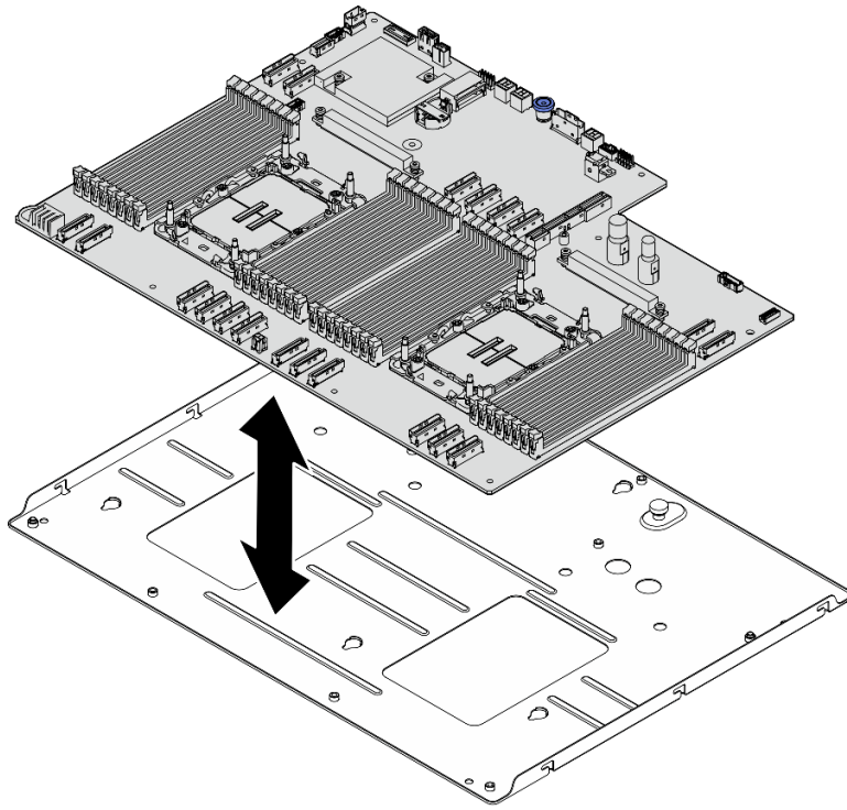
圖例 443. 拆卸主機板組件
