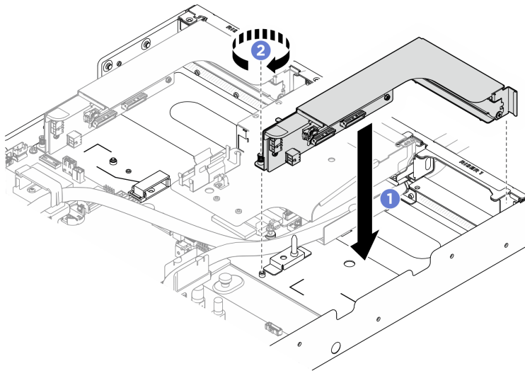
圖例 325. 將 PCIe 擴充卡組件安裝在插槽 1 中
