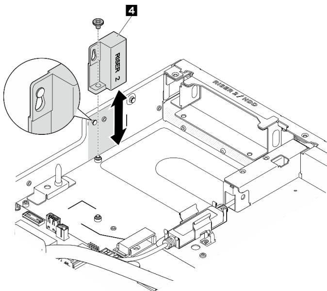
圖例 58. 從機箱卸下 DPU 空氣擋板
