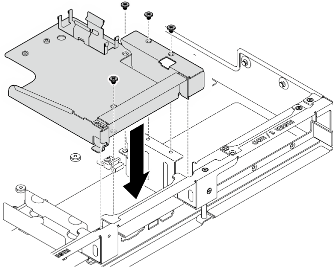
圖例 269. 安裝洩漏感應器模組托架
