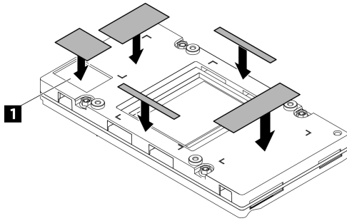
圖例 229. 更換 GPU 油灰墊
