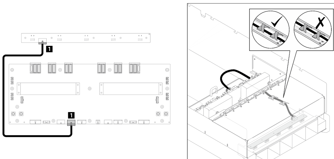
圖例 405. 後方風扇控制板纜線佈線
