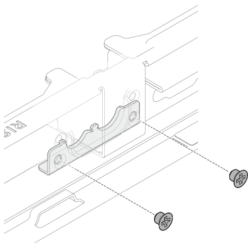
圖例 275. 卸下水管固定器
