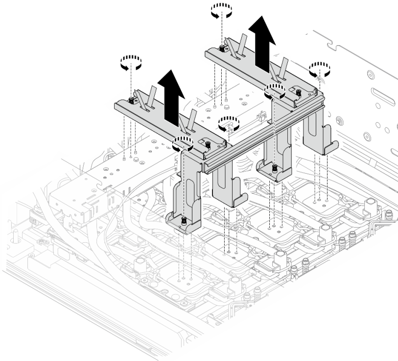
圖例 202. 卸下出貨托架
