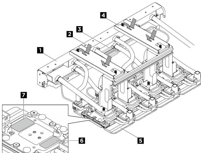
圖例 157. 前方 H100/H200 GPU 水冷板模組元件識別
