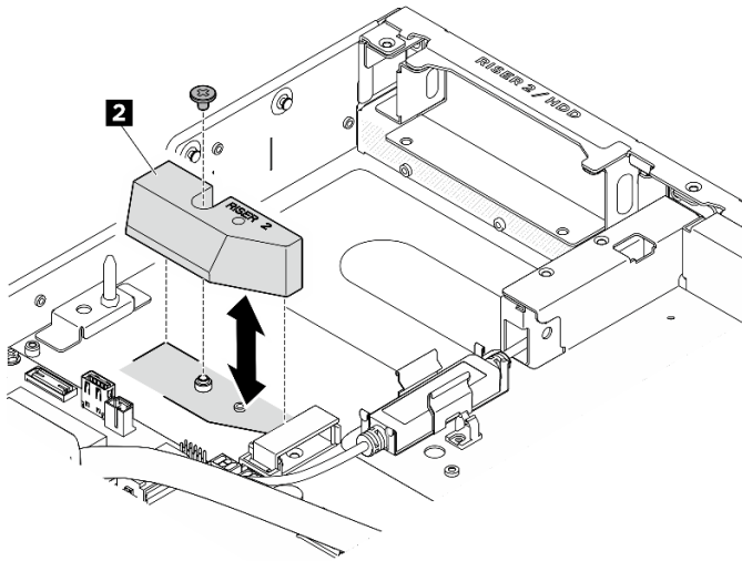
圖例 67. 將 DPU 空氣擋板安裝到機箱
