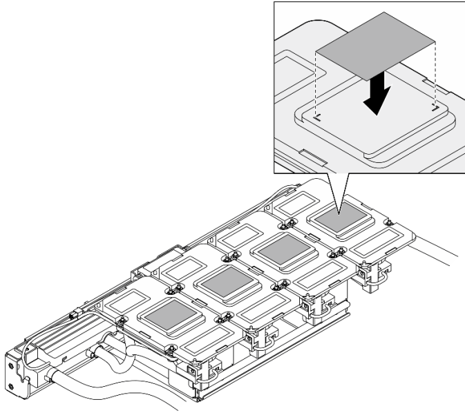
圖例 172. 貼附 PCM
