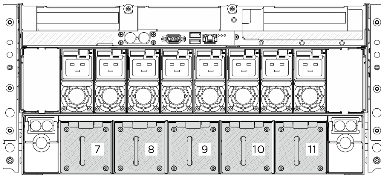
圖例 77. 後方風扇編號
