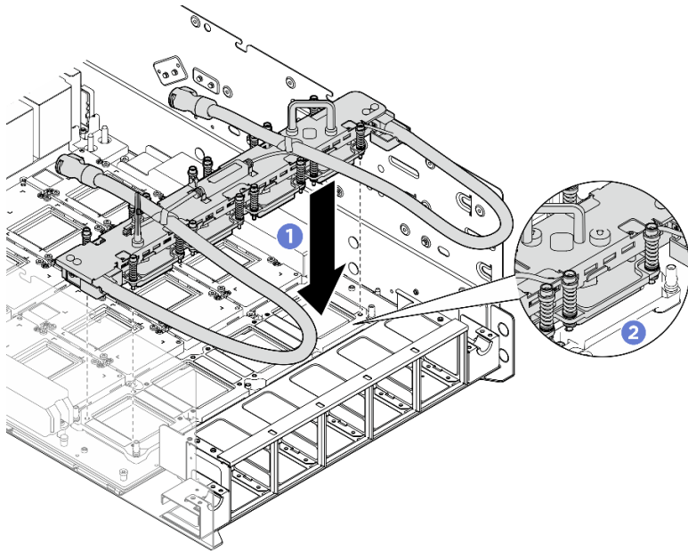
圖例 147. 安裝 NVSwitch 水冷板模組
