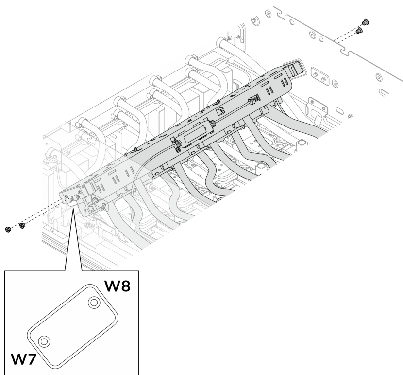
圖例 210. 安裝後方 H100/H200 GPU 水冷板模組歧管
