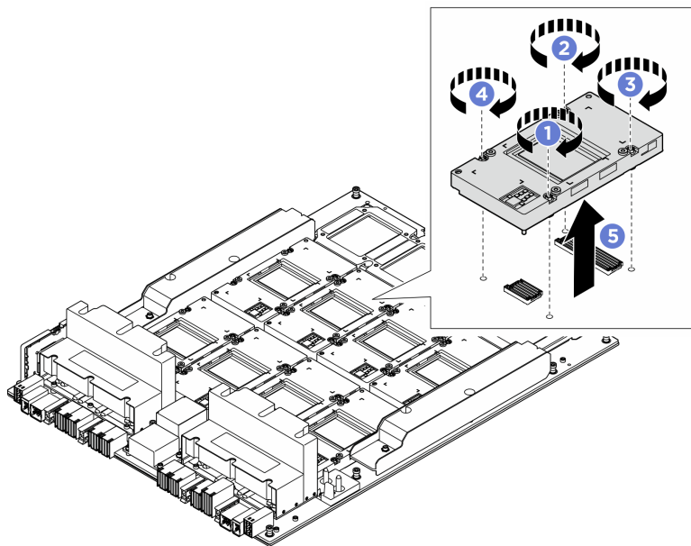
圖例 105. 卸下 GPU
