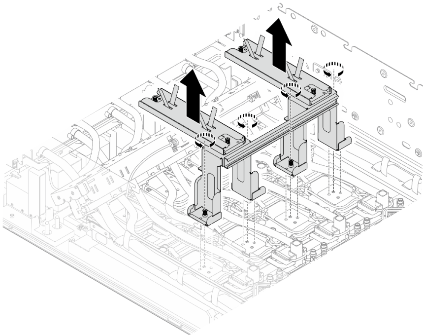
圖例 239. 卸下出貨托架
