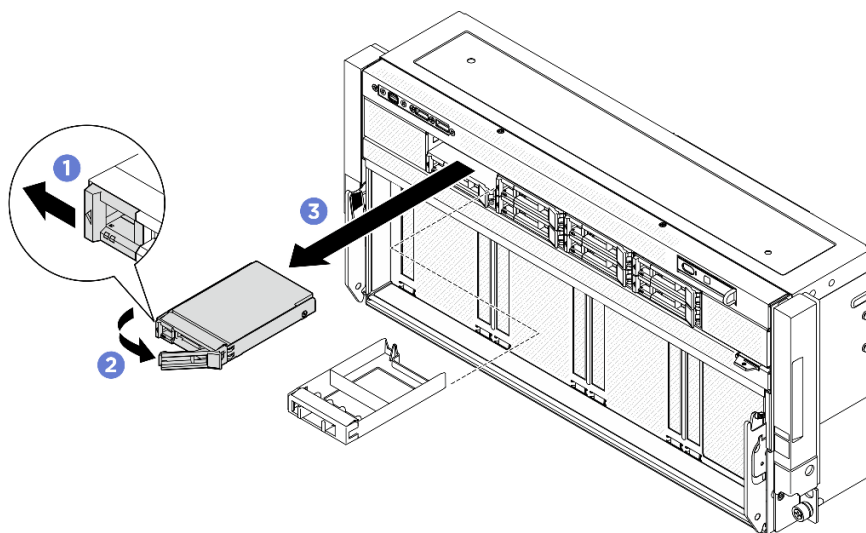
圖例 31. 卸下前方 2.5 吋熱抽換硬碟
