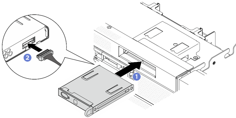
圖例 263. 安裝整合式診斷面板
