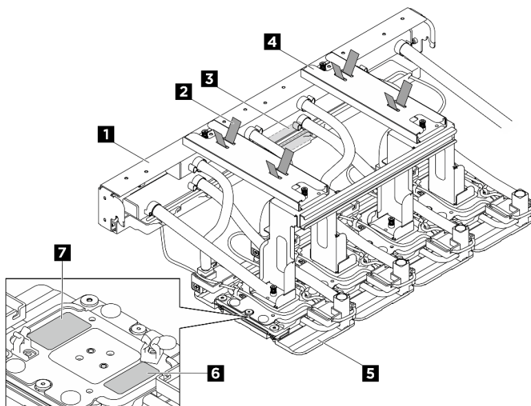
圖例 170. 前方 H100/H200 GPU 水冷板模組元件識別
