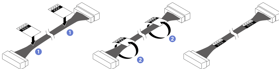
圖例 96. 黏貼標籤
