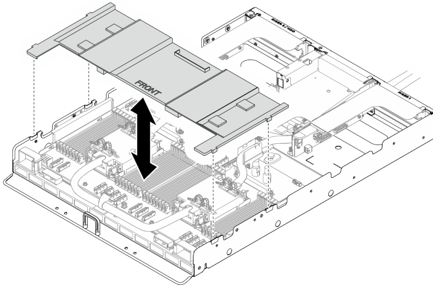
圖例 356. 安裝處理器空氣擋板
