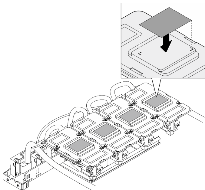
圖例 199. 貼附 PCM
