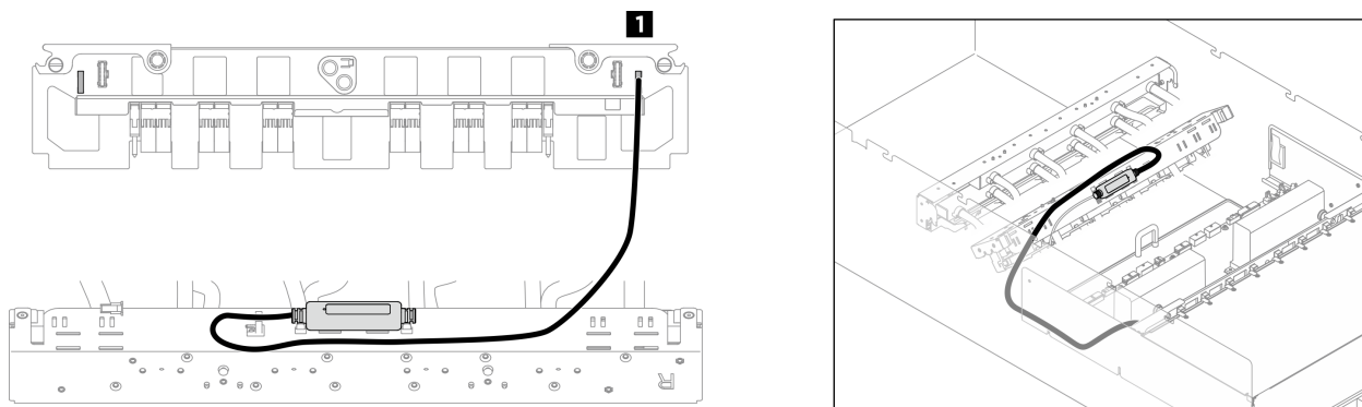
圖例 420. 後方 GPU 洩漏感應器模組纜線佈線
