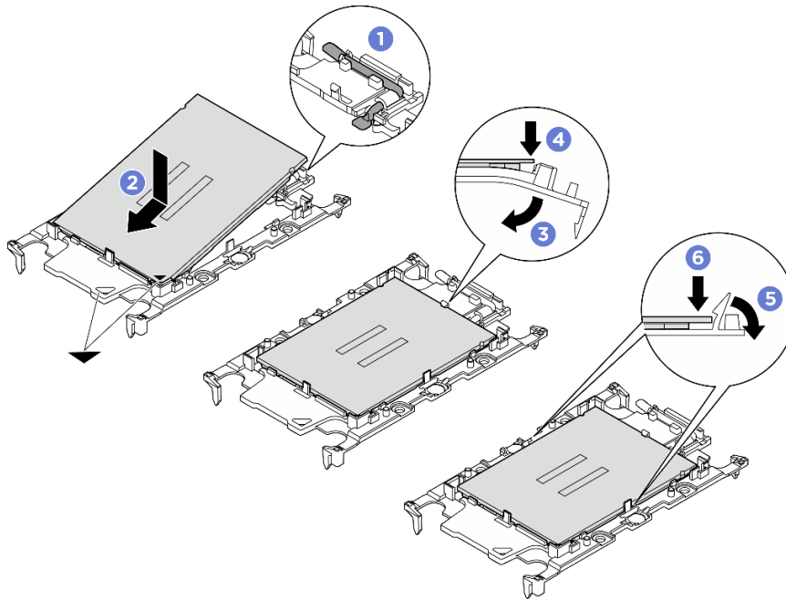
圖例 282. 安裝處理器支架
