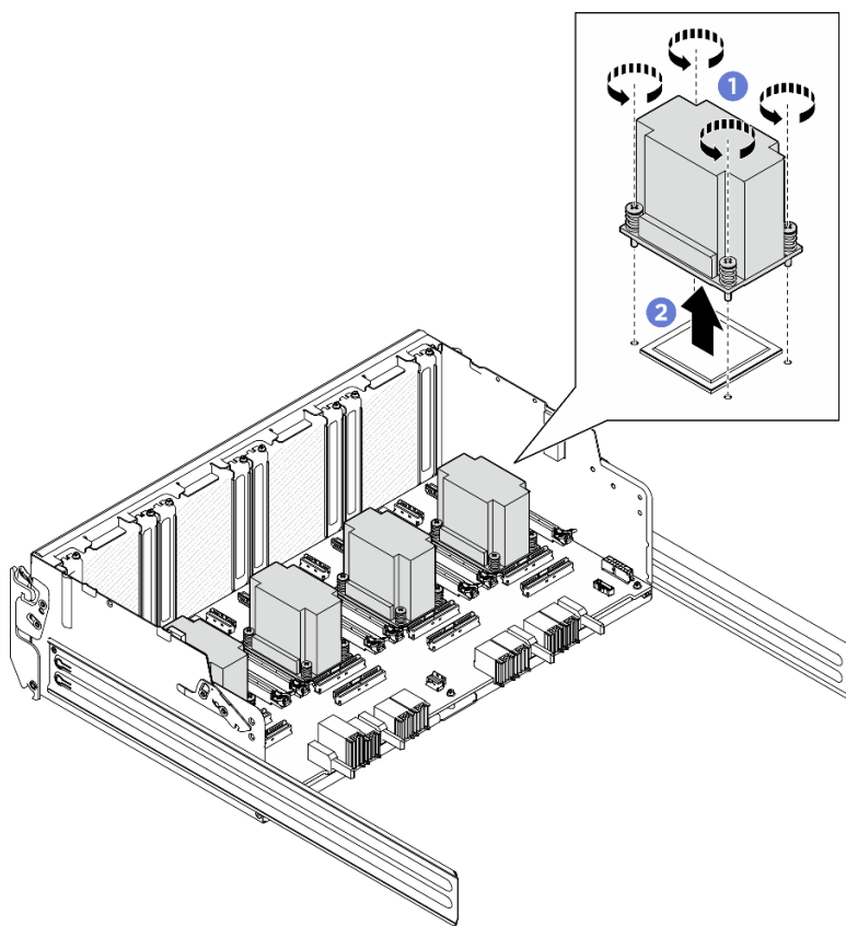
圖例 329. 卸下 PCIe 交換器板散熱槽
