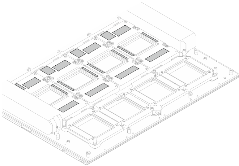
圖例 195. 清除 GPU 上的 PCM 和油灰墊
