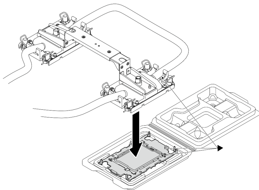
圖例 284. 組裝處理器與水冷板
