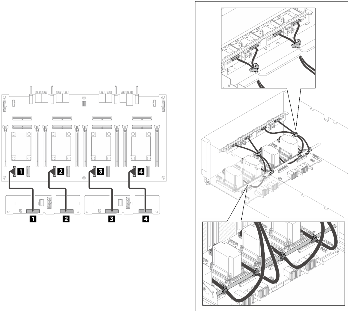
圖例 400. 前方 2.5 吋硬碟背板信號纜線佈線
