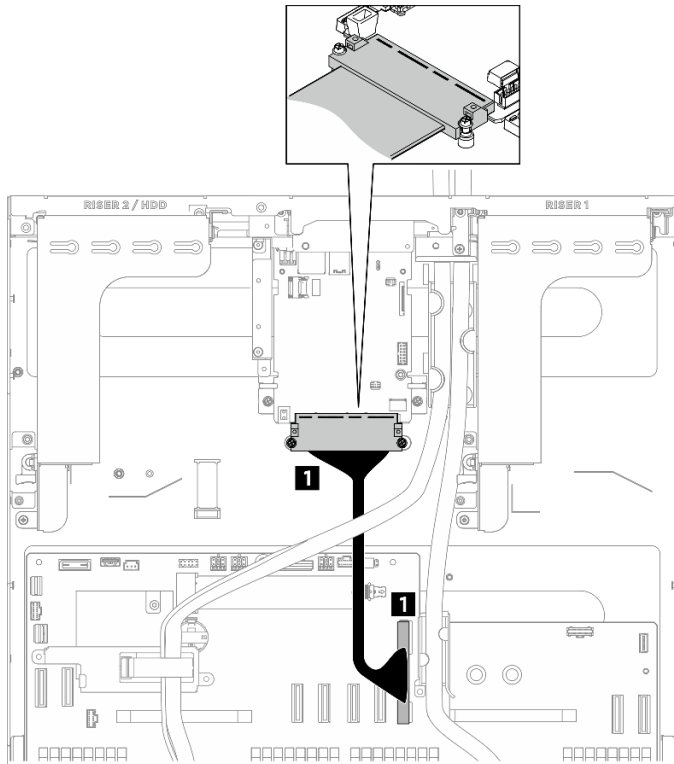
圖例 410. 系統 I/O 板纜線佈線
