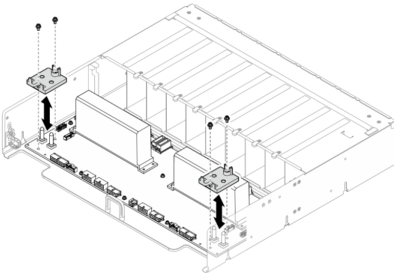
圖例 359. 卸下纜線固定器
