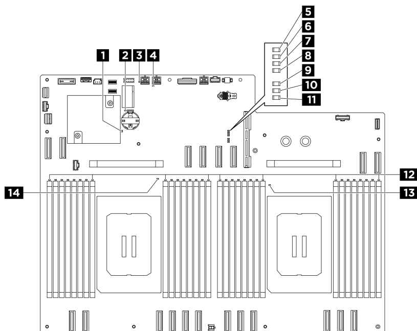
圖例 433. 主機板 LED
