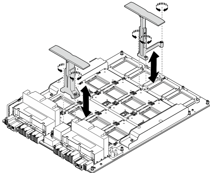
圖例 104. 卸下把手
