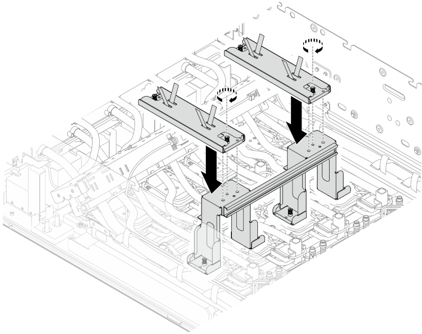
圖例 238. 安裝把手
