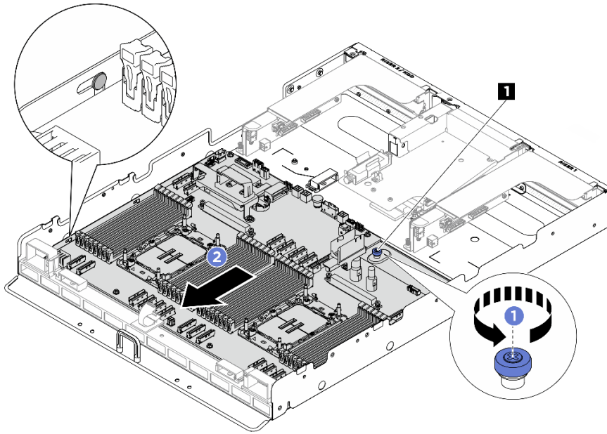
圖例 383. 鬆開主機板
