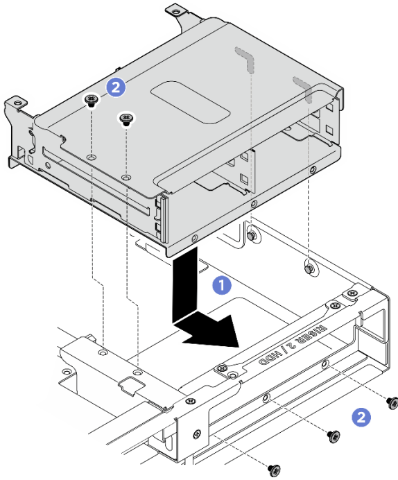
圖例 379. 安裝背面框架
