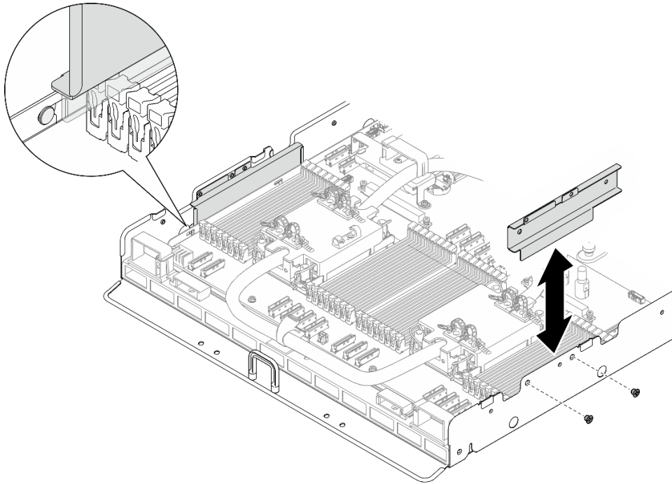
圖例 382. 卸下纜線導件
