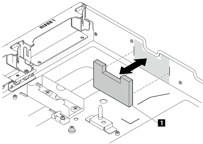
圖例 51. 從機箱卸下 DPU 空氣擋板
