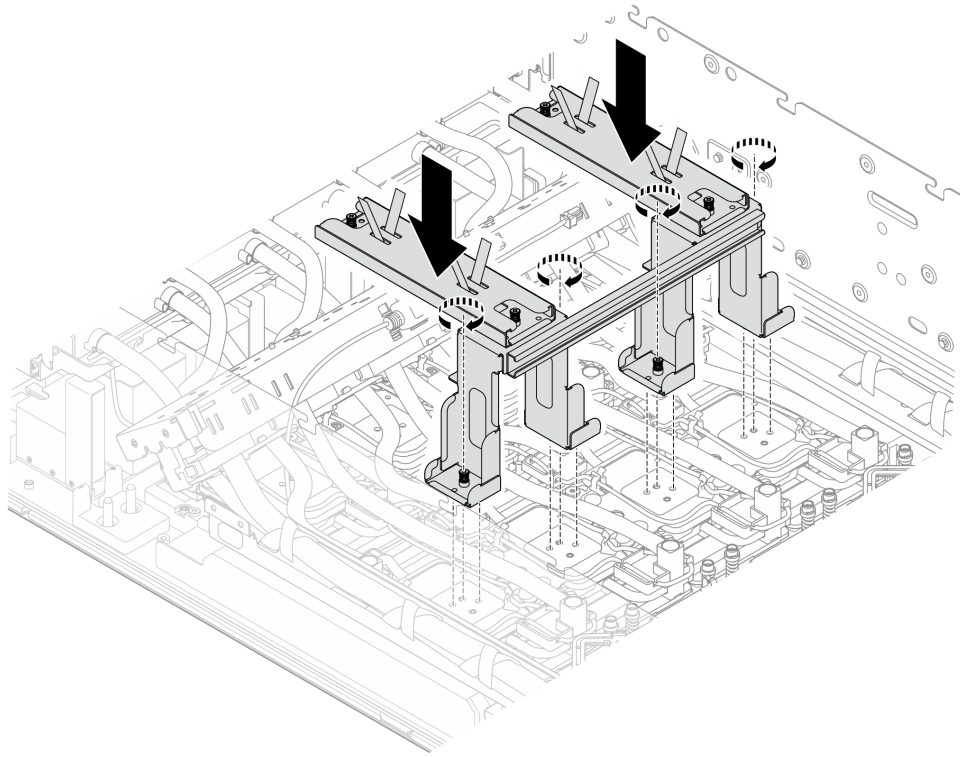
圖例 213. 將出貨托架安裝到後方 GPU 水冷板
