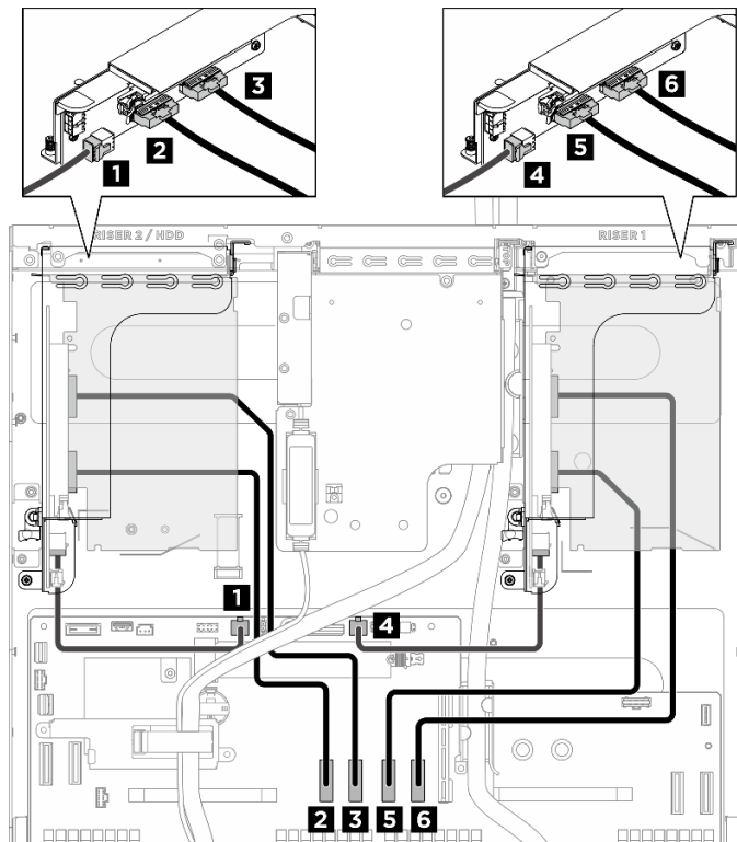
圖例 416. PCIe 擴充卡纜線佈線
