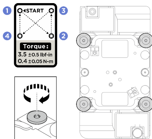
圖例 258. 安裝 GPU 水冷板
