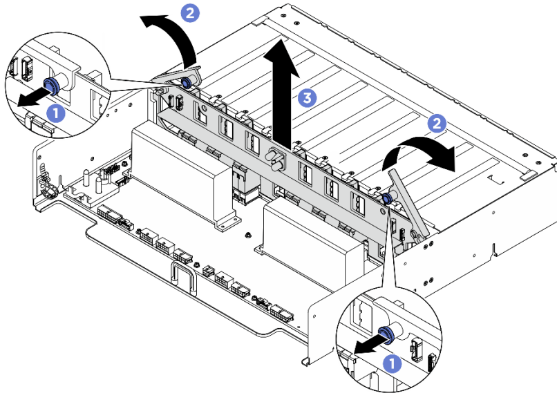
圖例 365. 卸下 PSU 轉插卡
