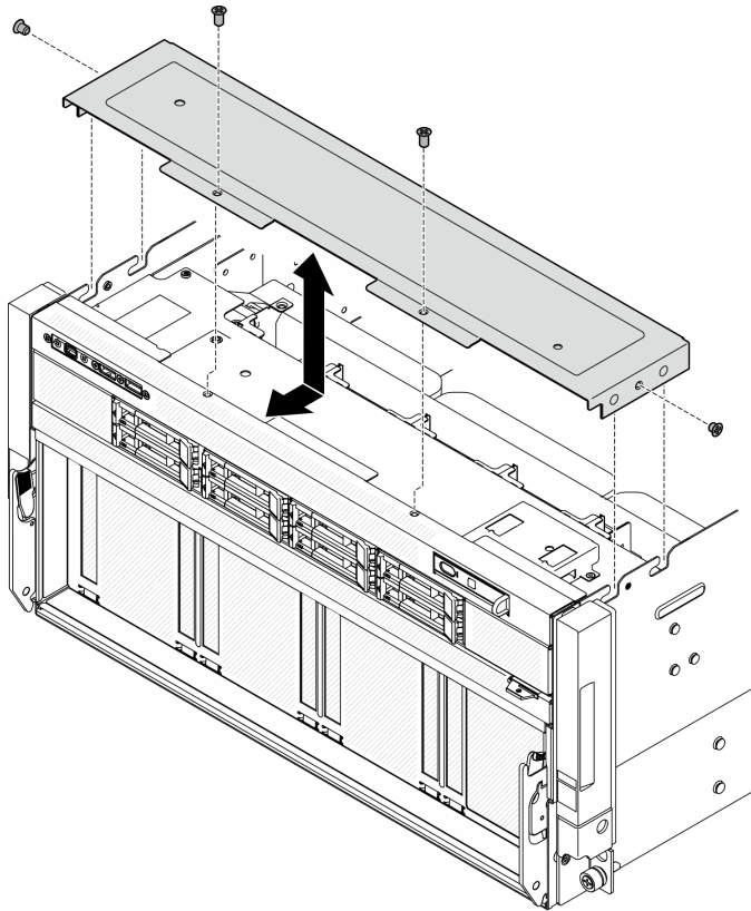
圖例 266. 安裝 I/O 蓋板
