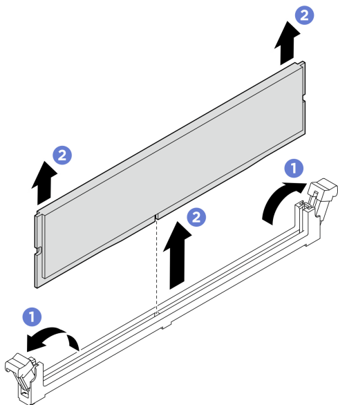
圖例 305. 卸下記憶體模組
