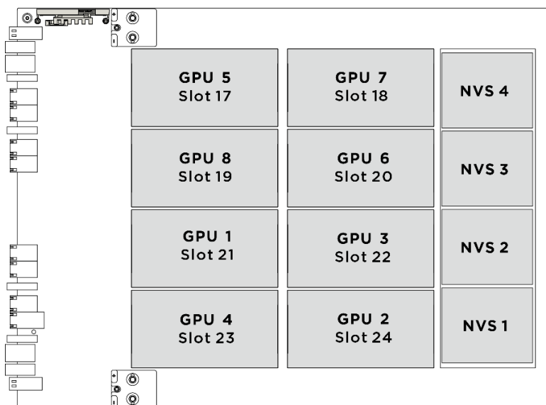
圖例 97. GPU 編號
