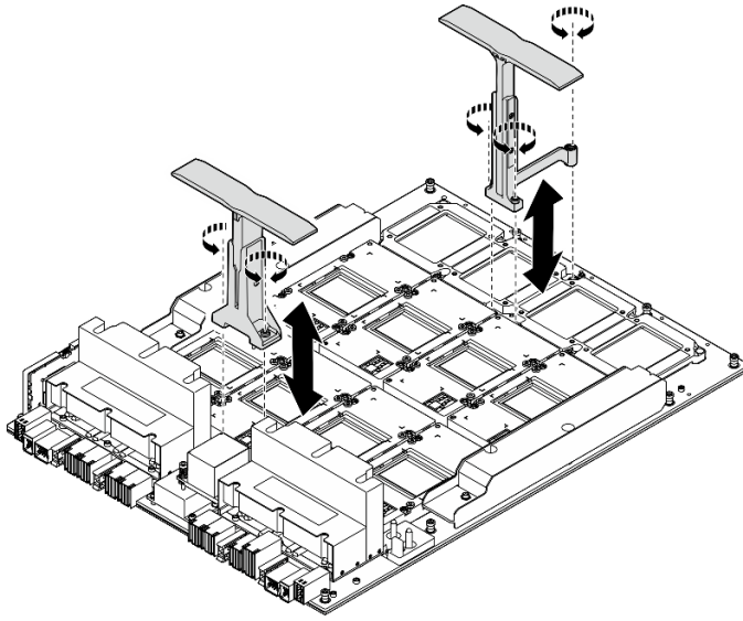
圖例 111. 卸下把手
