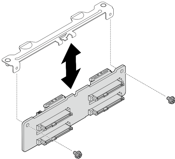
圖例 374. 安裝後方 2.5 吋硬碟背板
