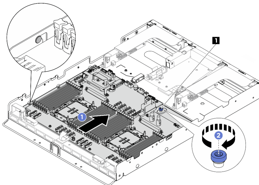
圖例 386. 固定主機板
