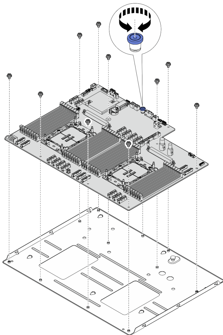
圖例 442. 卸下元件
