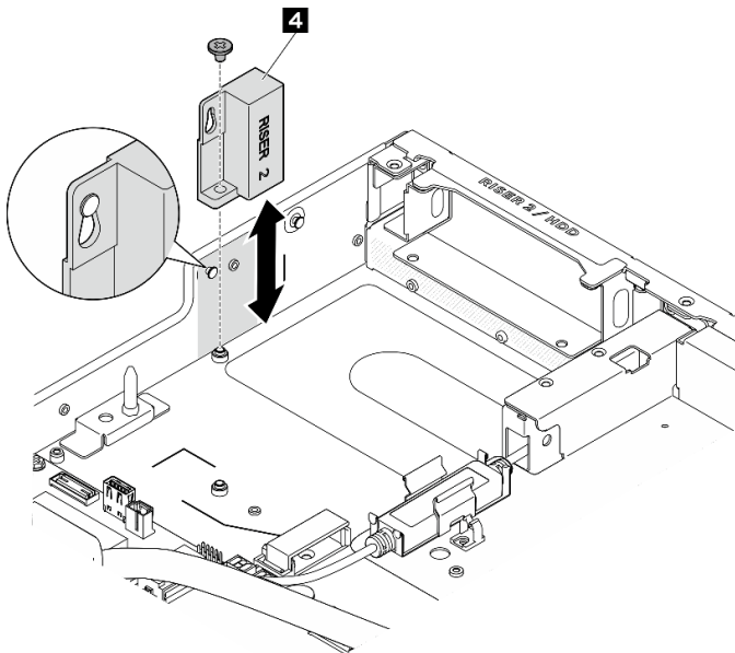
圖例 69. 將 DPU 空氣擋板安裝到機箱
