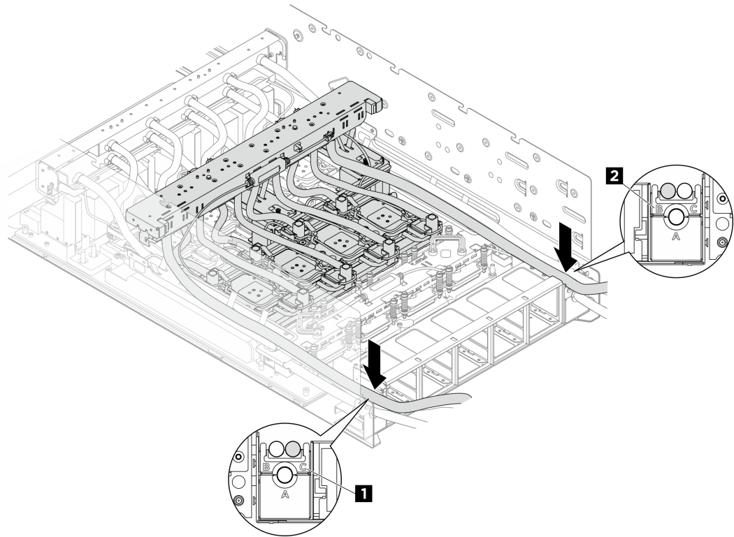
圖例 208. 將軟管放在水管固定器上
