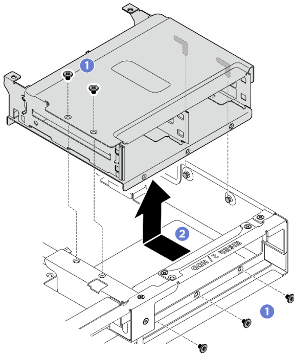
圖例 367. 卸下背面框架
