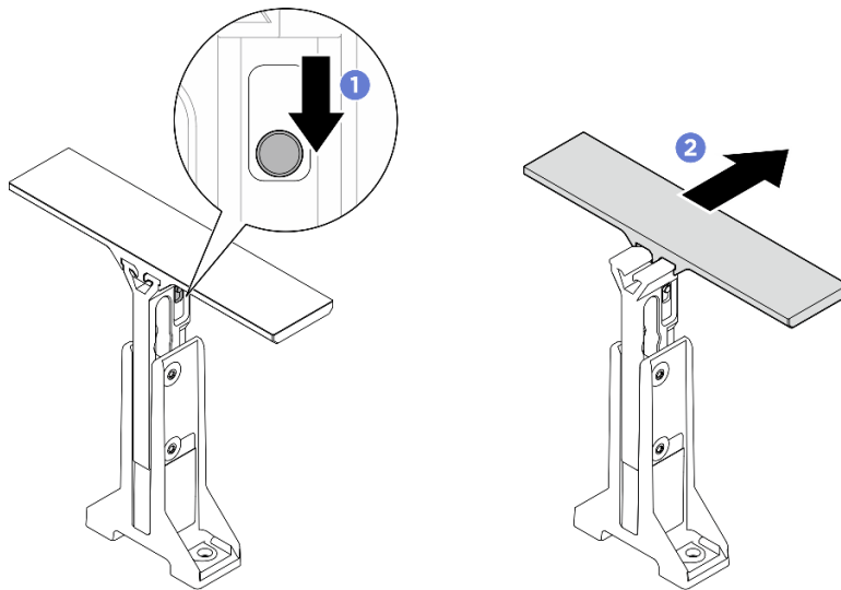
圖例 123. 調整把手
