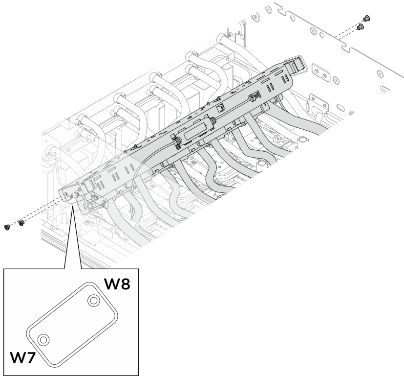
圖例 215. 卸下後方 H100/H200 GPU 水冷板模組歧管
