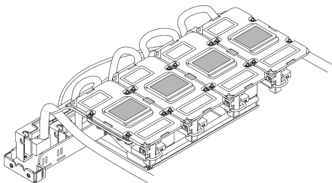
圖例 196. 擦掉水冷板上的 PCM 和油灰墊
