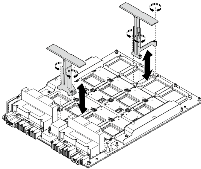
圖例 102. 安裝把手
