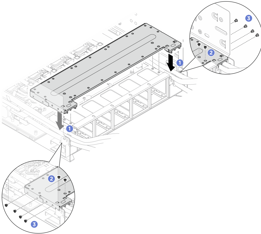
圖例 185. 安裝後方風扇機盒支撐托架
