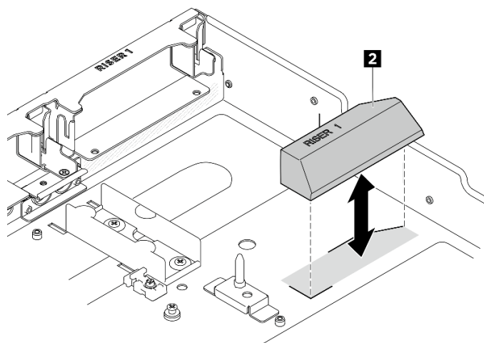
圖例 62. 將 DPU 空氣擋板安裝到機箱
