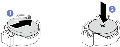
圖例 49. CMOS 電池安裝
