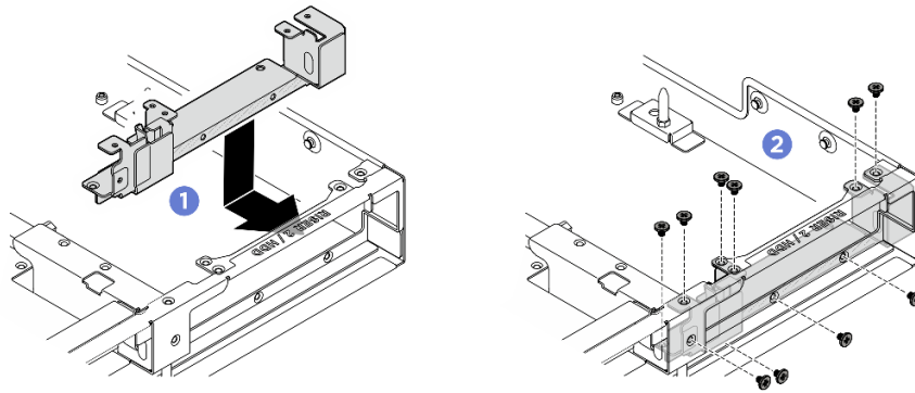
圖例 326. 安裝背面擴充卡支撐托架
