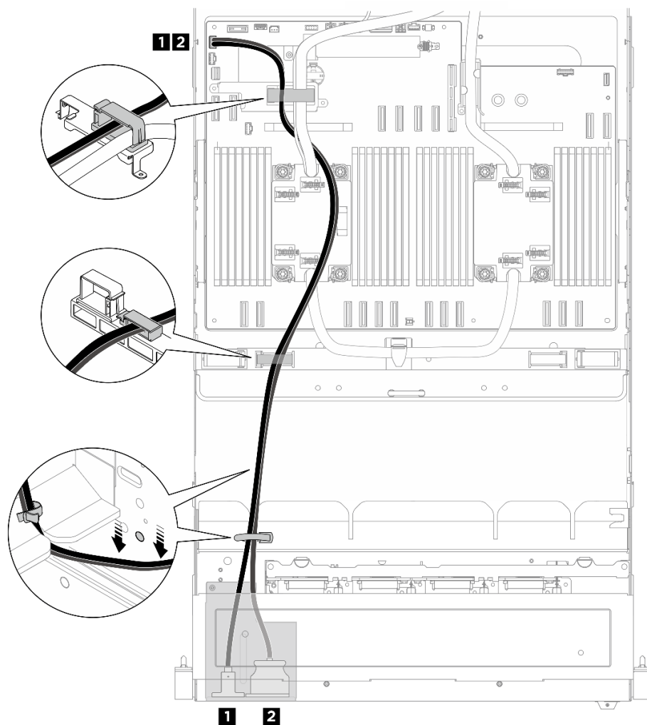
圖例 407. 正面 I/O 模組纜線佈線
