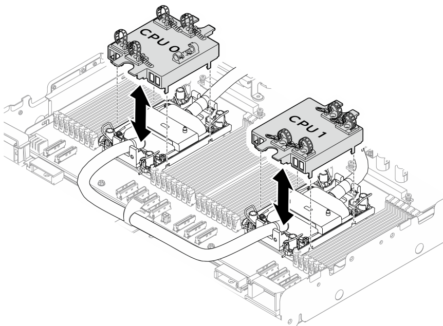
圖例 288. 安裝水冷板蓋
