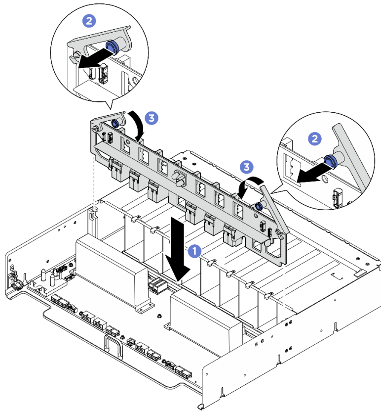
圖例 363. 安裝 PSU 轉插卡
