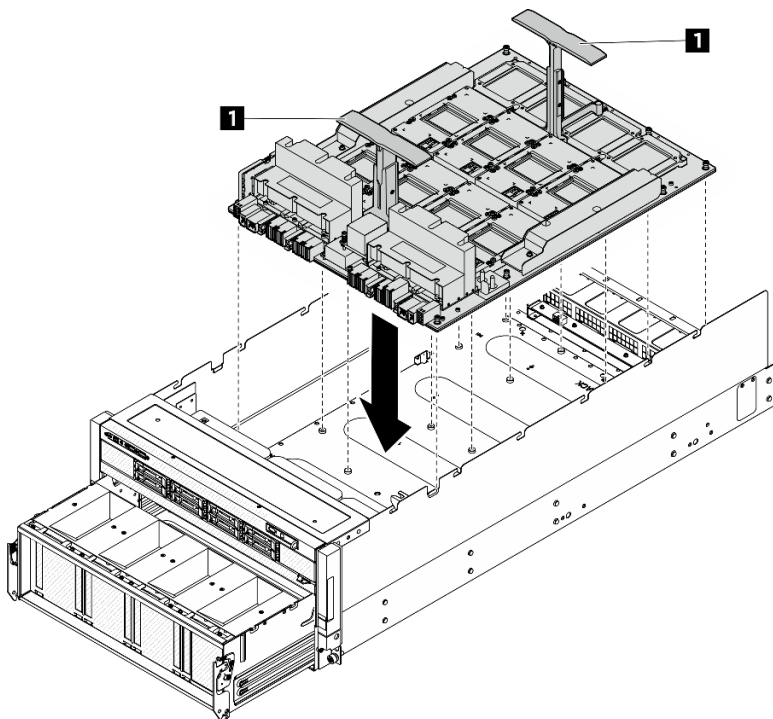
圖例 109. 安裝 GPU 複合體
