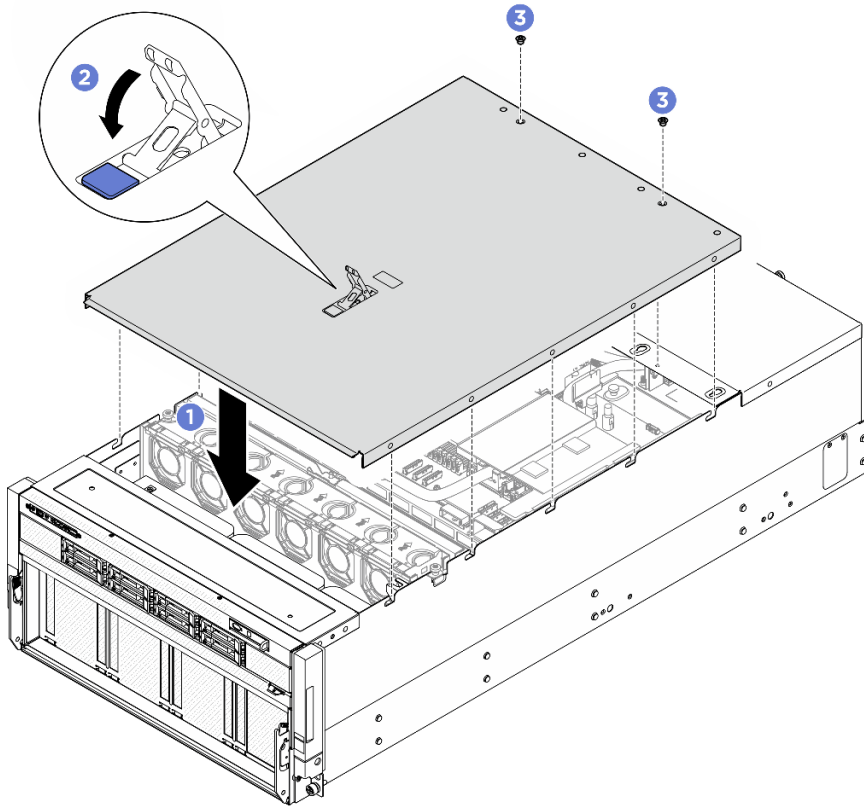
圖例 26. 安裝前方上蓋
