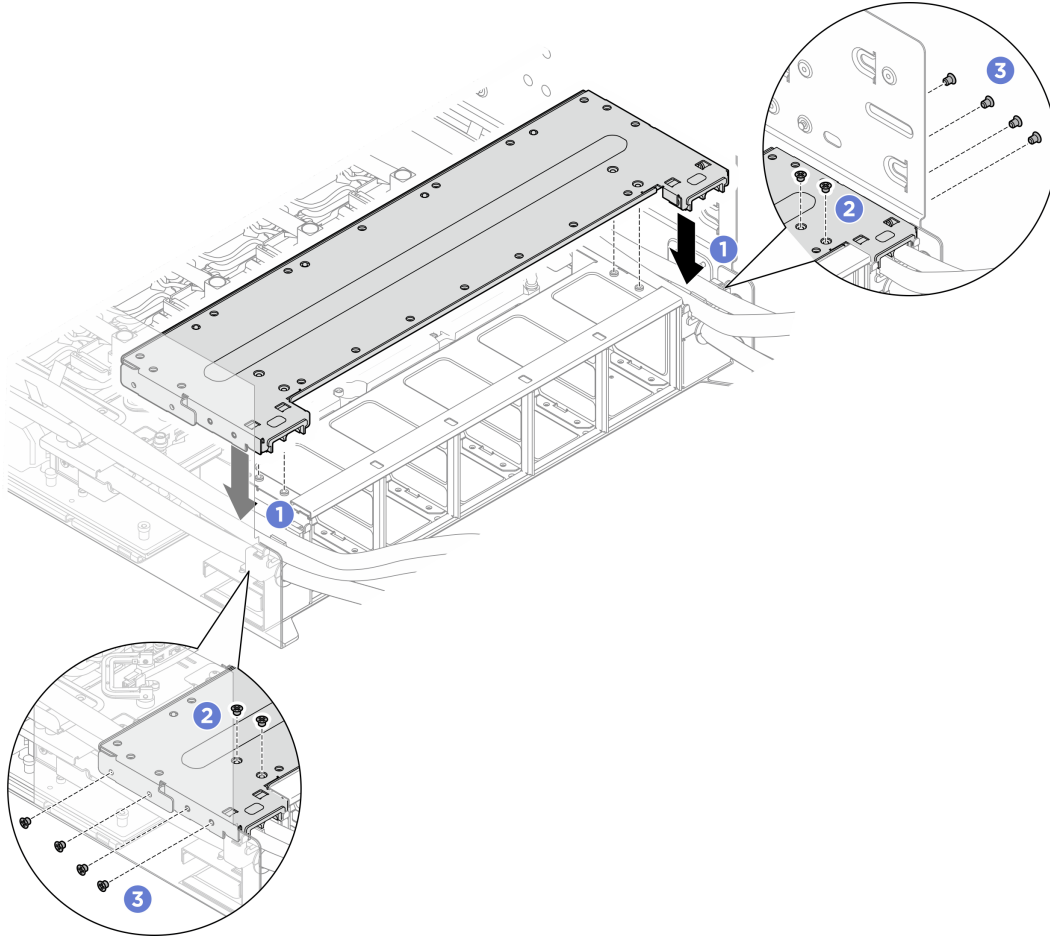
圖例 211. 安裝後方風扇機盒支撐托架
