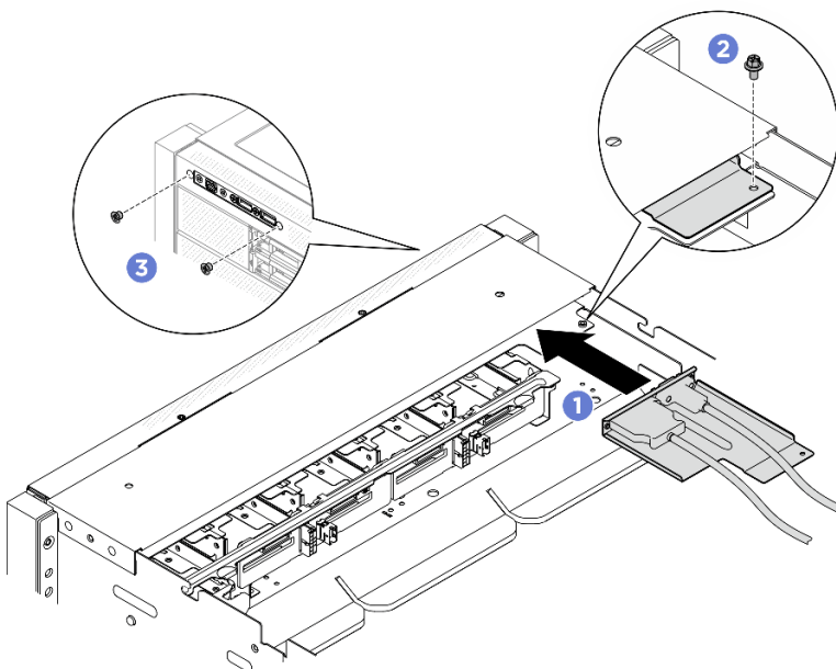
圖例 95. 安裝正面 I/O 模組
