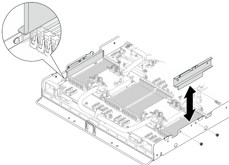
圖例 387. 安裝纜線導件
