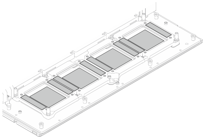
圖例 143. 清除 NVSwitch 上的 PCM 和油灰墊
