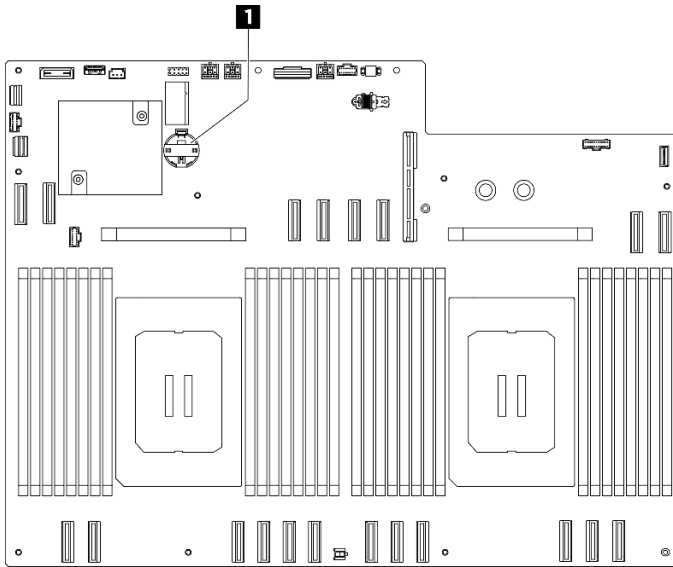
圖例 46. CMOS 電池位置
