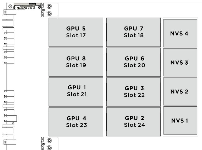
圖例 133. GPU 編號
