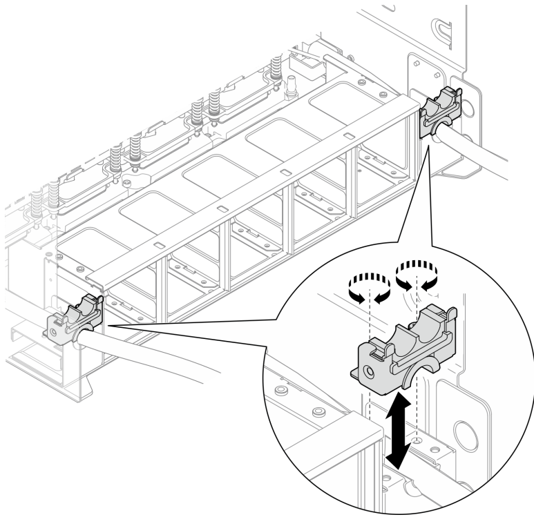
圖例 137. 卸下水管固定器 B/C
