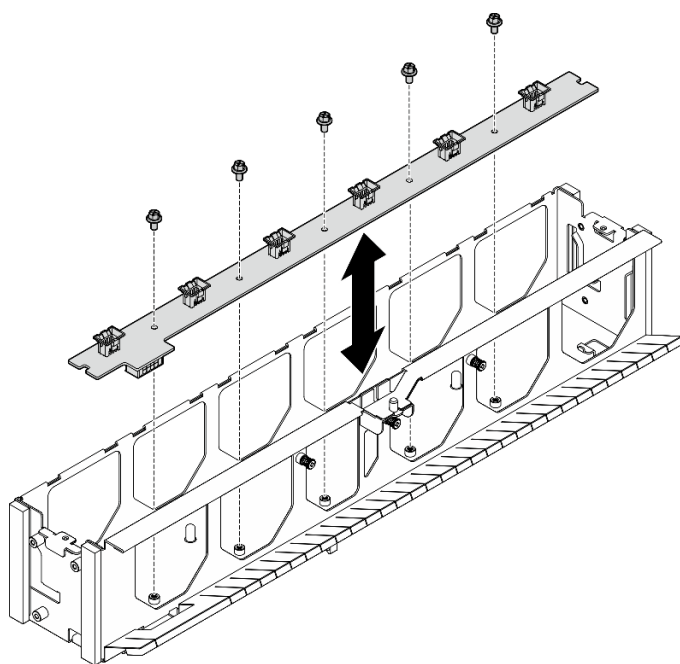
圖例 84. 安裝前方風扇控制板
