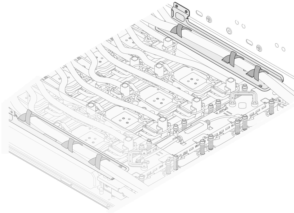
圖例 138. 將軟管和纜線從軟管束帶上鬆開
