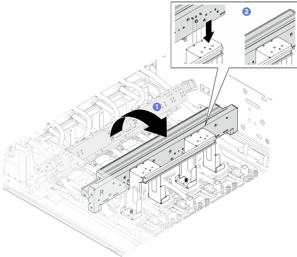
圖例 216. 重新放置後方 GPU 水冷板模組歧管
