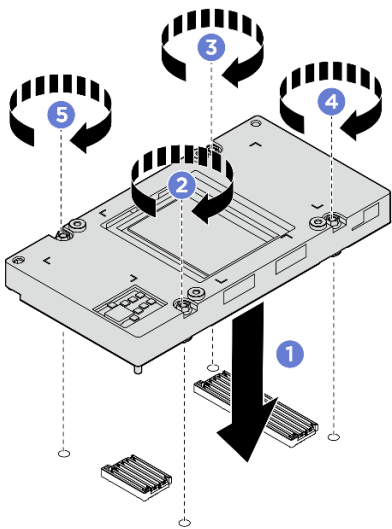
圖例 227. 安裝 GPU
