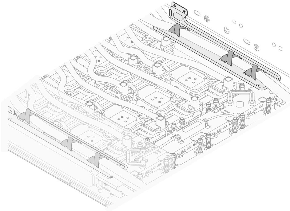
圖例 154. 將軟管和纜線放在軟管導管上
