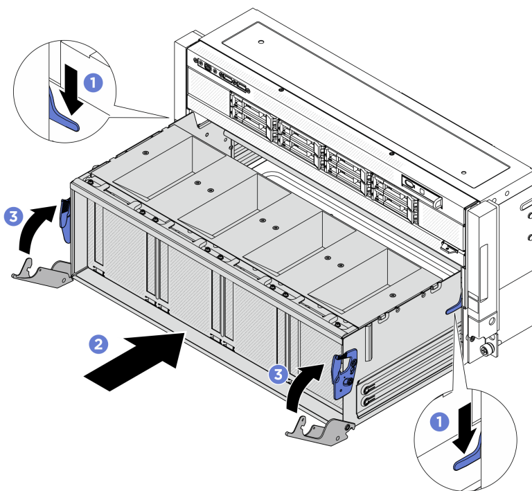
圖例 340. 安裝 PCIe 交換器滑動箱
