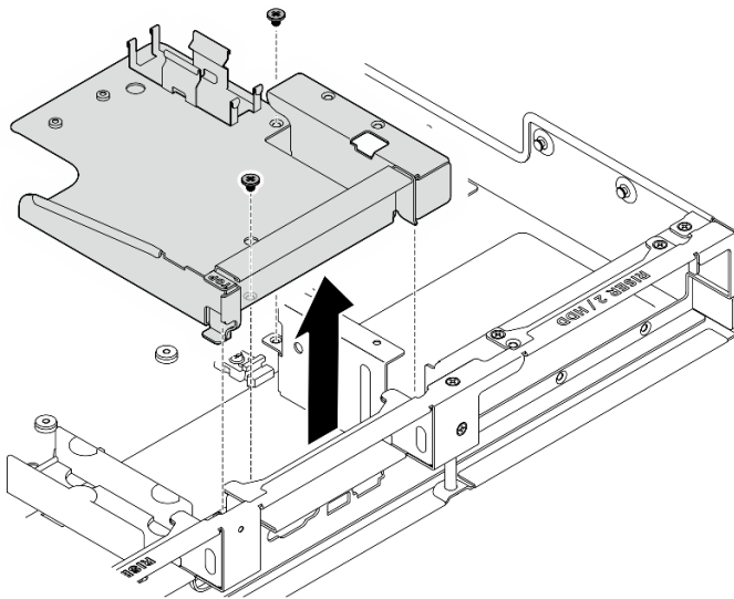
圖例 368. 卸下洩漏感應器模組托架
