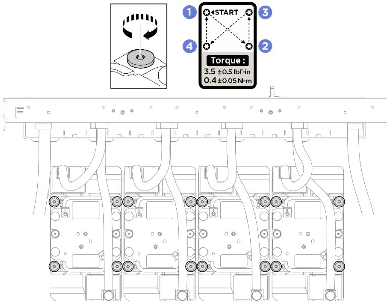
圖例 179. 安裝 GPU 水冷板
