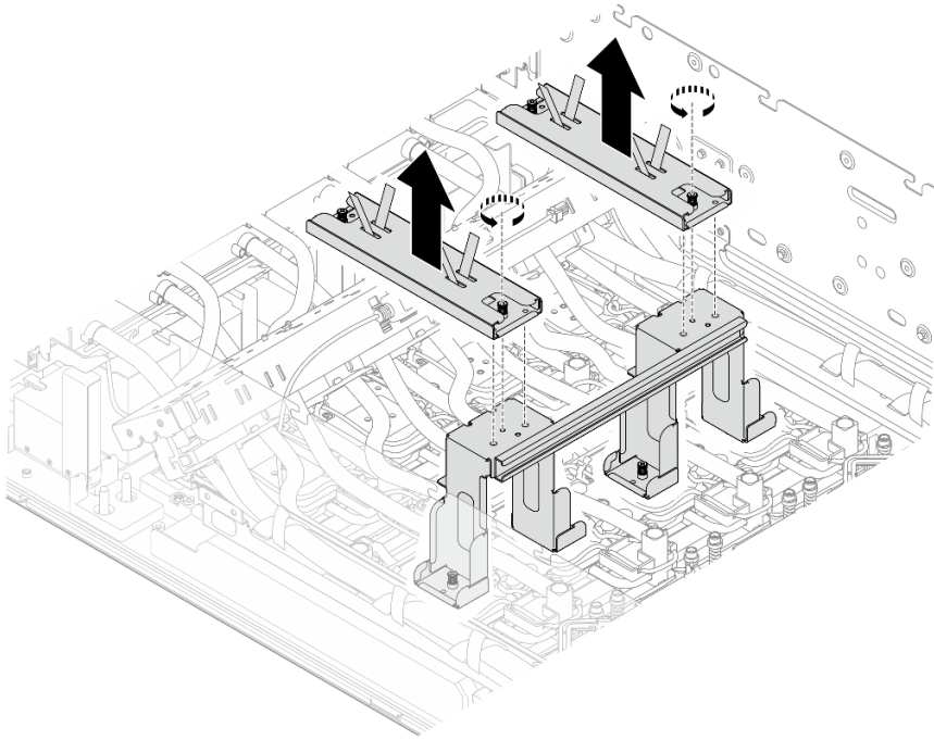
圖例 214. 從出貨托架卸下把手
