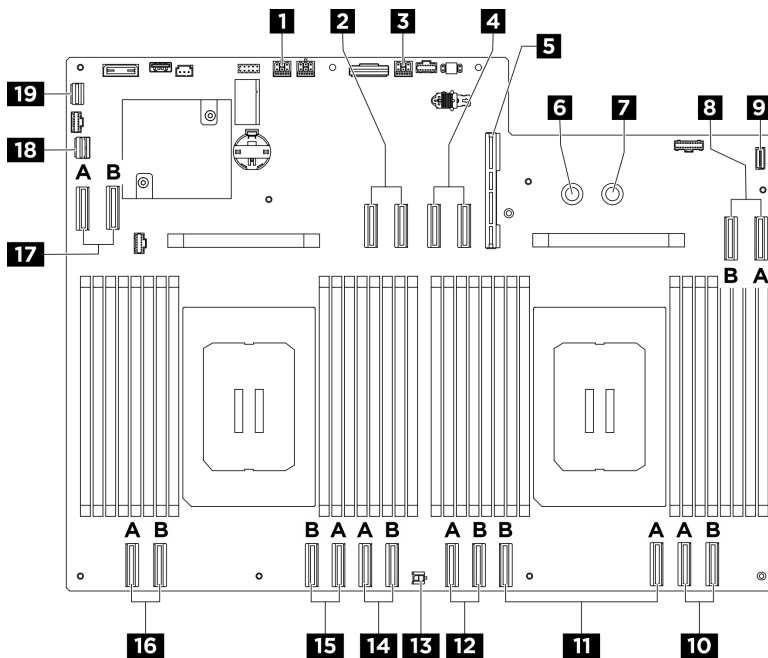
圖例 399. 用於纜線佈線的主機板接頭
