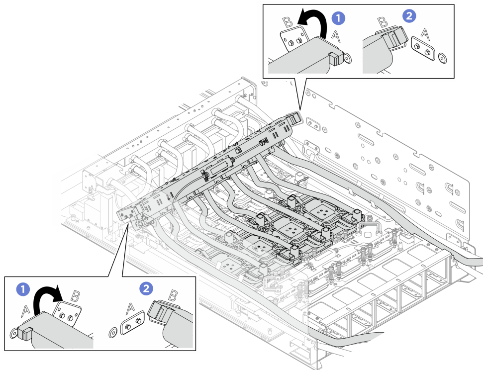
圖例 183. 重新安裝後方 H100/H200 GPU 水冷板模組歧管
