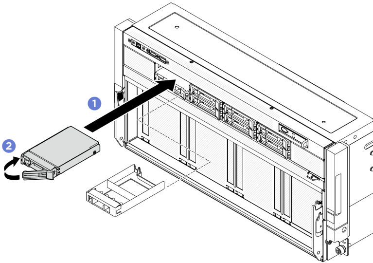
圖例 35. 安裝正面 2.5 吋熱抽換硬碟
