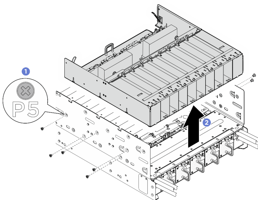
圖例 341. 卸下電源複合體
