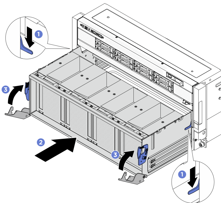
圖例 315. 安裝 PCIe 交換器滑動箱
