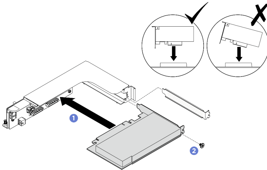
圖例 317. 安裝背面 PCIe 配接卡
