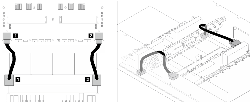
圖例 406. GPU 基板纜線佈線
