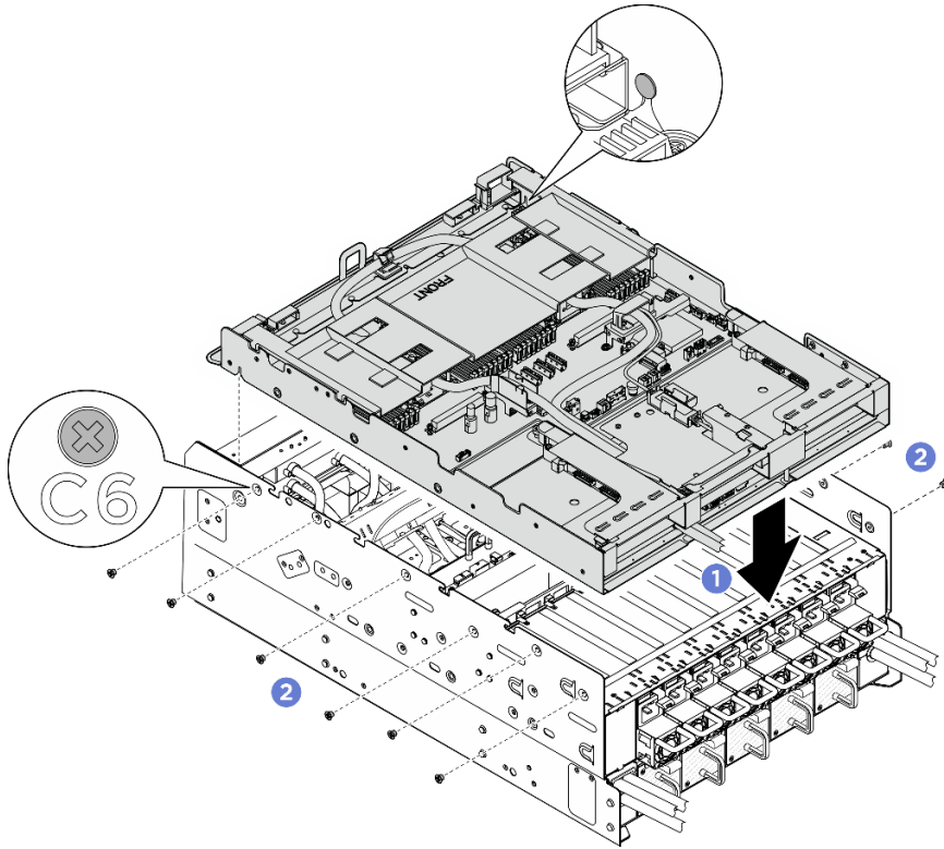
圖例 45. 安裝 CPU 複合體
