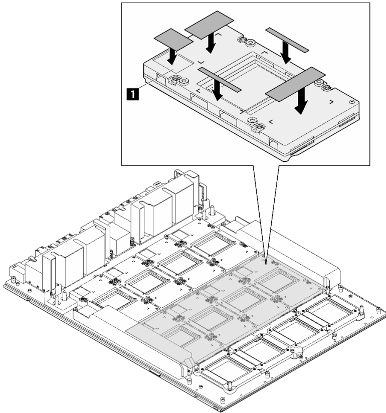
圖例 200. 更換 GPU 油灰墊
