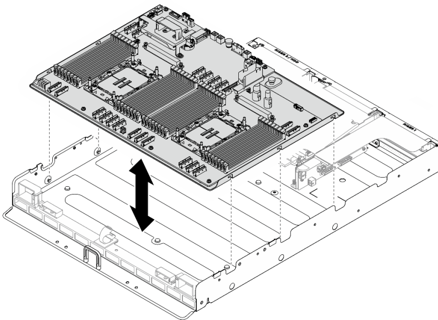
圖例 385. 安裝主機板
