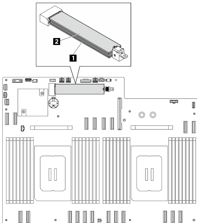
圖例 301. M.2 硬碟插槽
