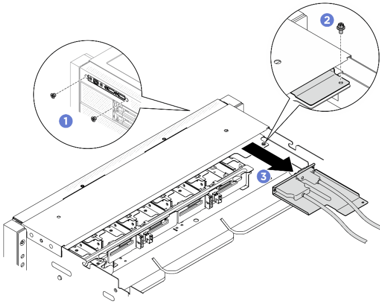
圖例 92. 卸下正面 I/O 模組
