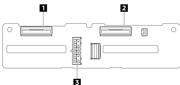
圖例 392. 2.5 吋硬碟背板接頭
