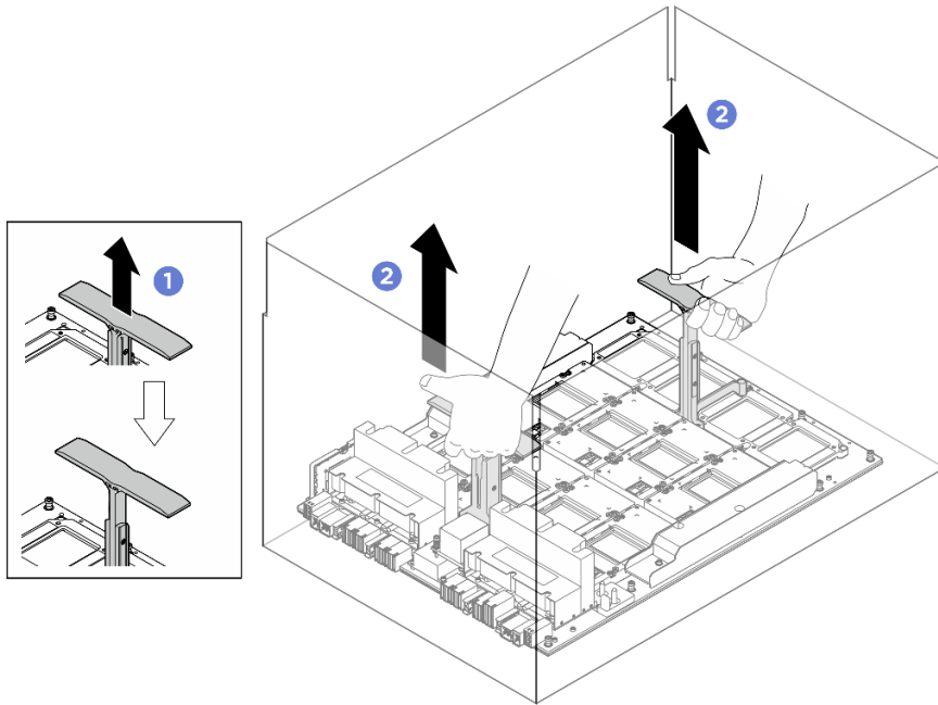
圖例 121. 從包裝盒中取出 GPU 複合體
