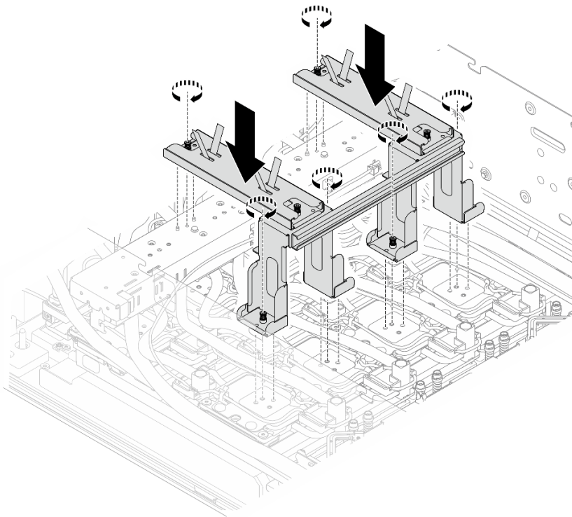
圖例 193. 安裝出貨托架
