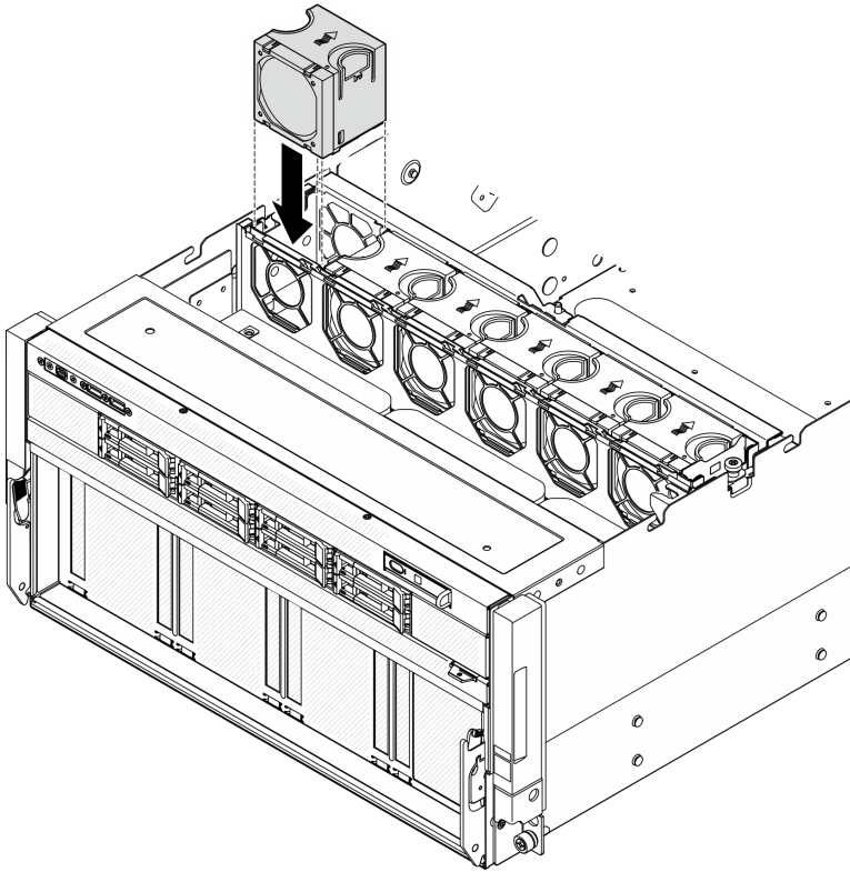
圖例 76. 前方風扇安裝
