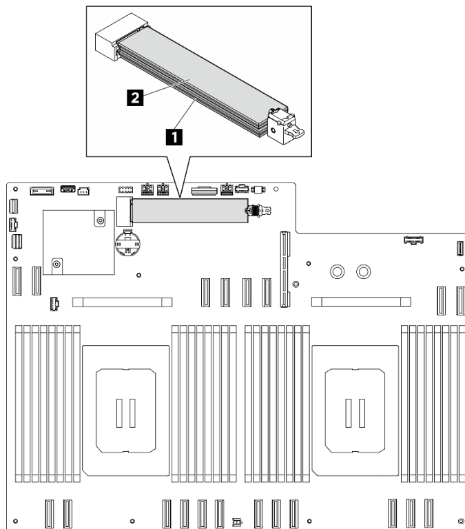
圖例 297. M.2 硬碟插槽
