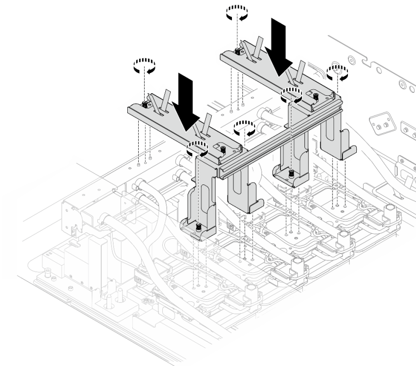
圖例 163. 安裝出貨托架
