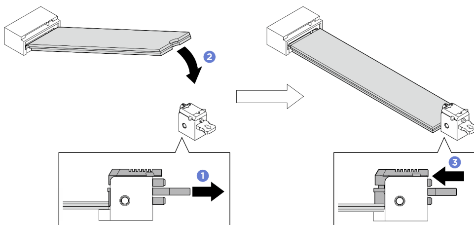
圖例 302. 安裝下方 M.2 硬碟
