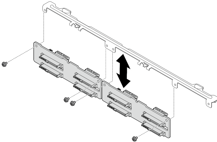
圖例 41. 安裝前方 2.5 吋硬碟背板
