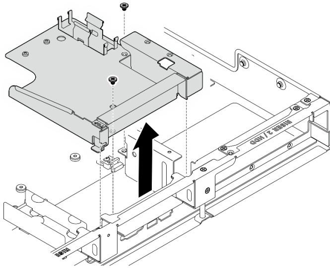
圖例 268. 卸下洩漏感應器模組托架
