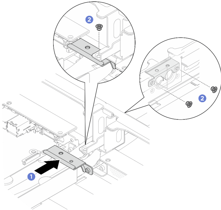
圖例 294. 安裝軟管蓋
