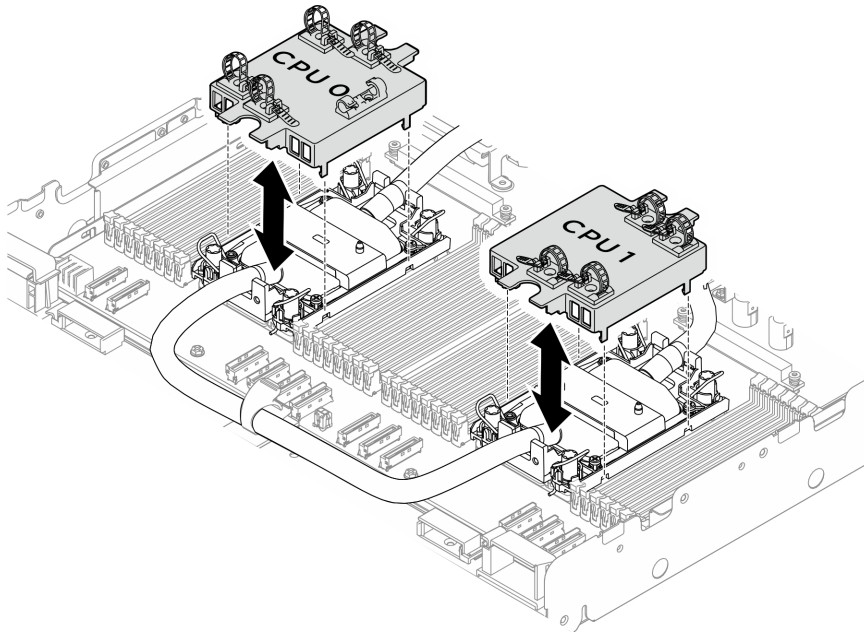
圖例 278. 卸下水冷板上蓋
