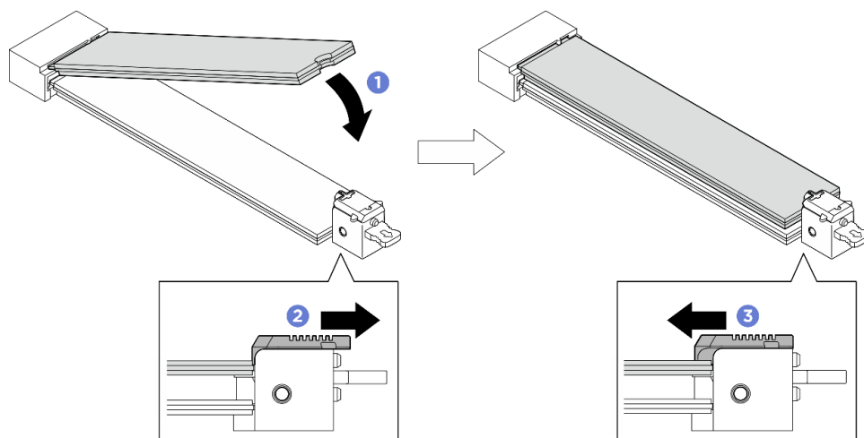
圖例 303. 安裝上方 M.2 硬碟
