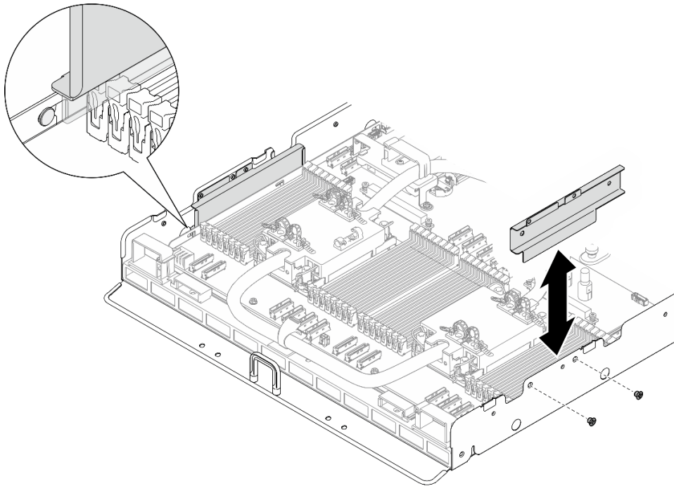
圖例 436. 卸下纜線導件
