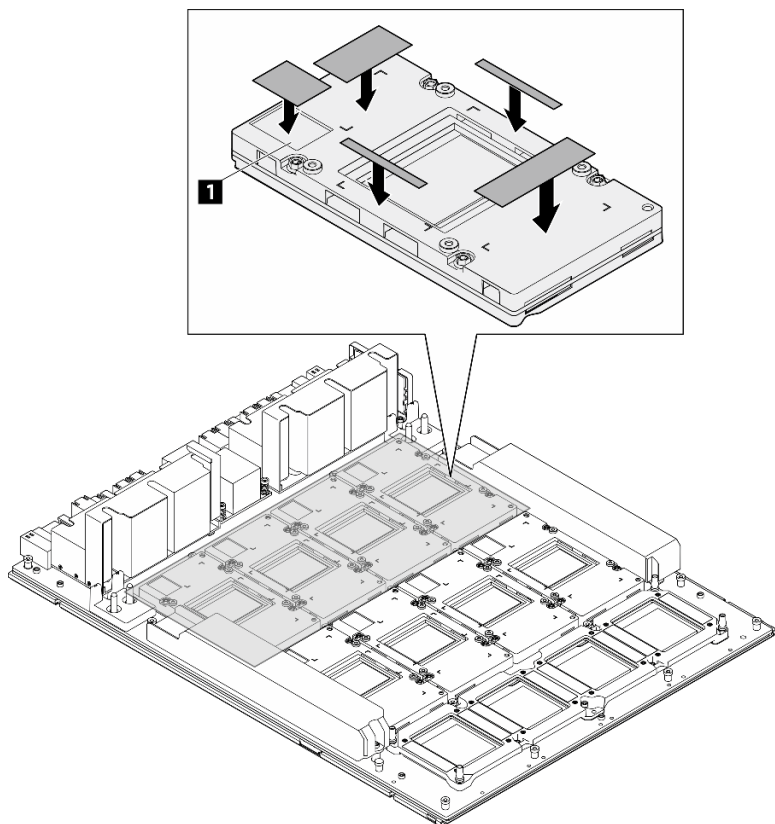
圖例 173. 更換 GPU 油灰墊
