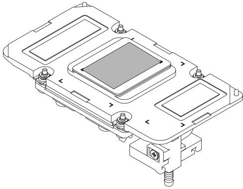
圖例 247. 擦掉水冷板上的 PCM 和油灰墊
