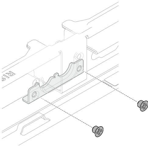
圖例 293. 固定水管固定器
