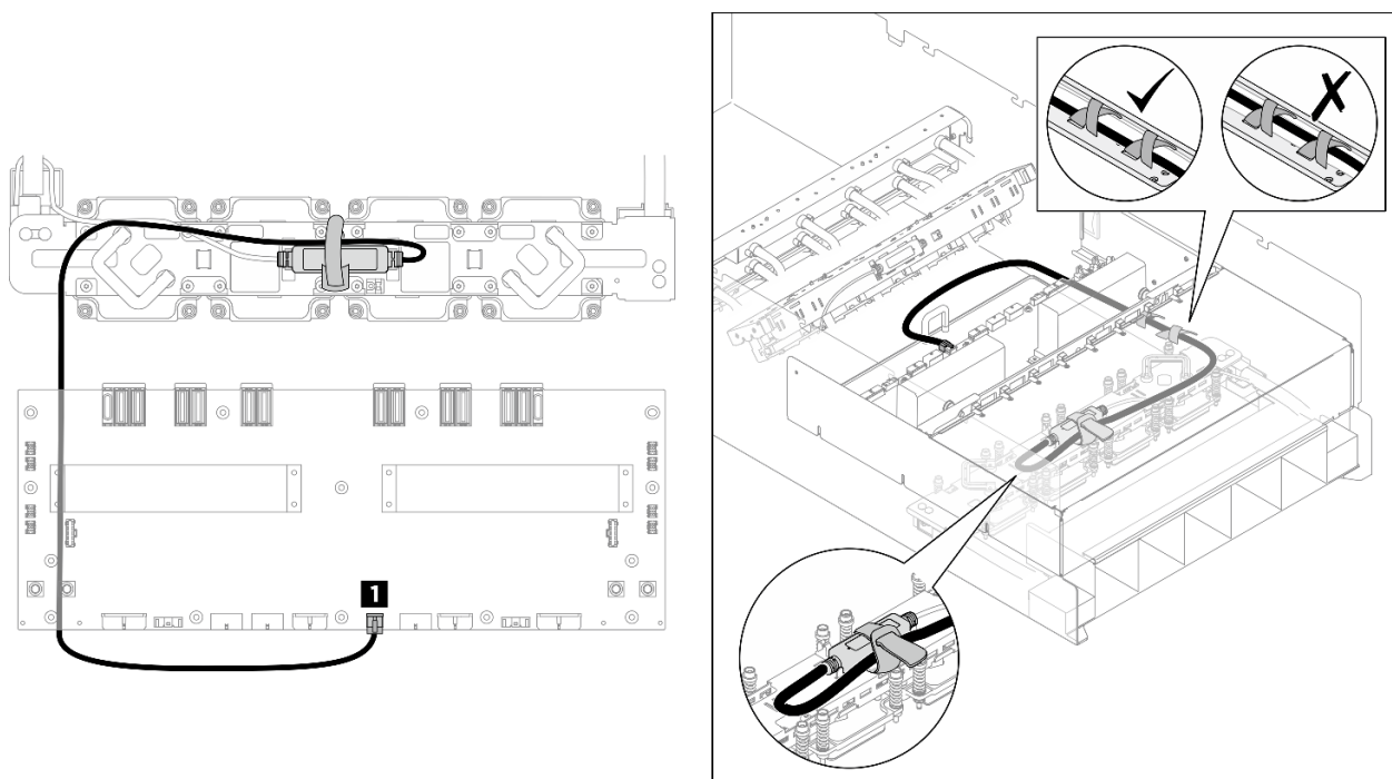
圖例 418. NVSwitch 洩漏感應器模組纜線佈線
