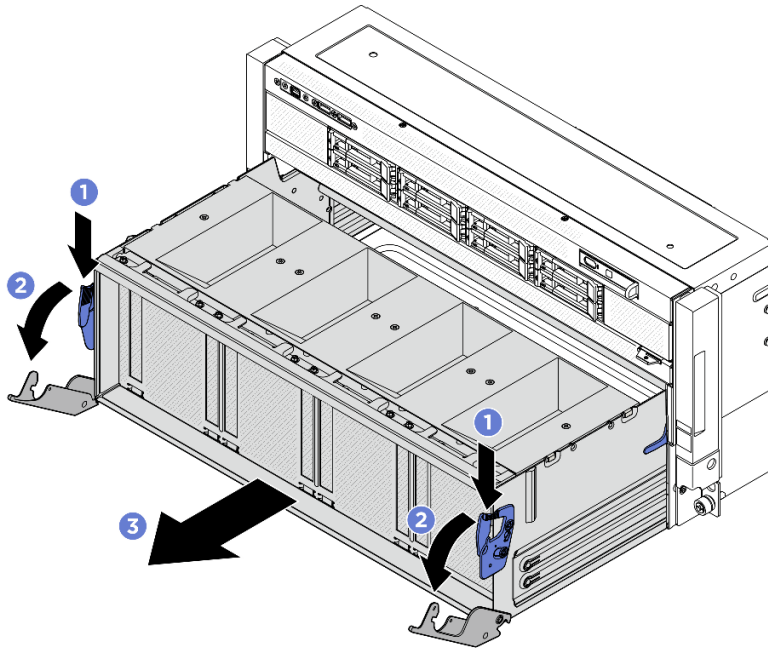
圖例 128. 將 PCIe 交換器滑動箱從停止位置卸下
