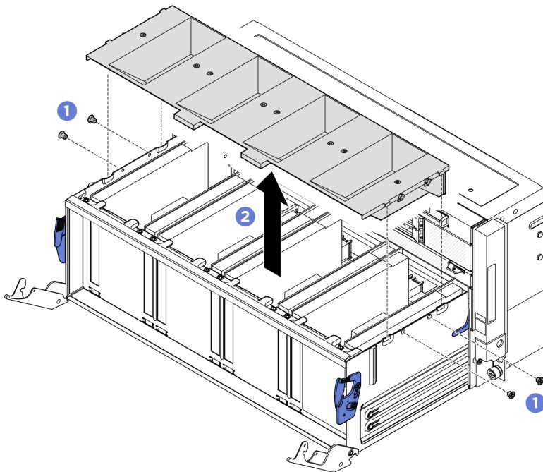
圖例 335. 卸下空氣擋板
