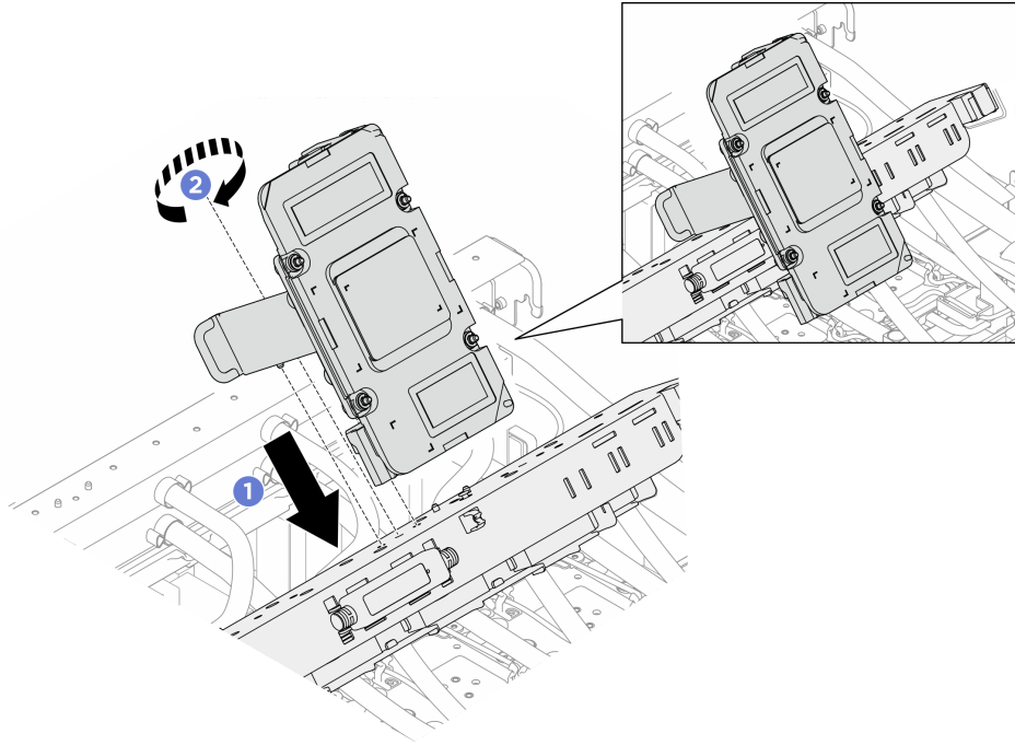
圖例 244. 安裝維修托架和 GPU 水冷板組件
