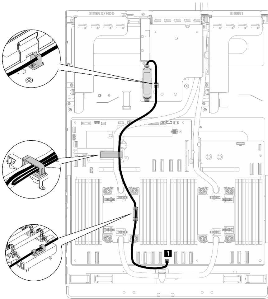
圖例 421. DWCM 洩漏感應器模組纜線佈線
