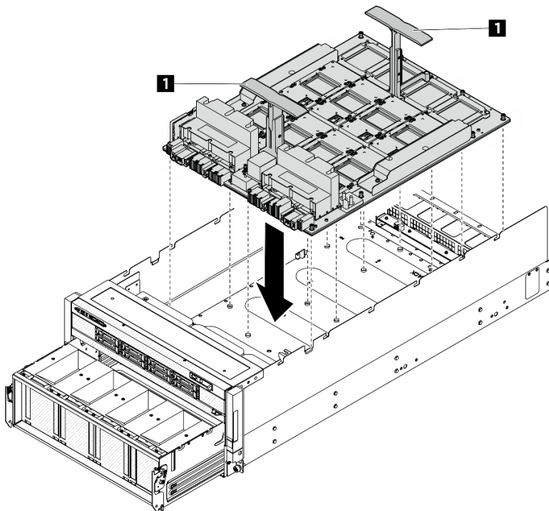
圖例 122. 安裝 GPU 複合體
