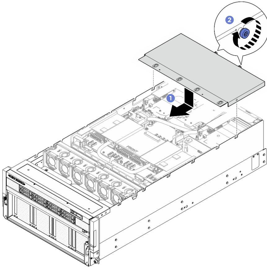
圖例 28. 安裝後方上蓋
