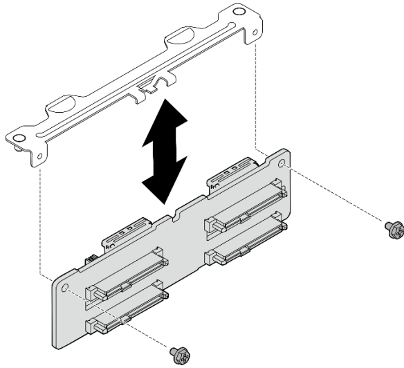
圖例 372. 卸下後方 2.5 吋硬碟背板
