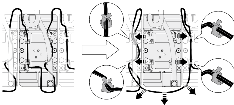
圖例 217. 移除洩漏感應器模組纜線
