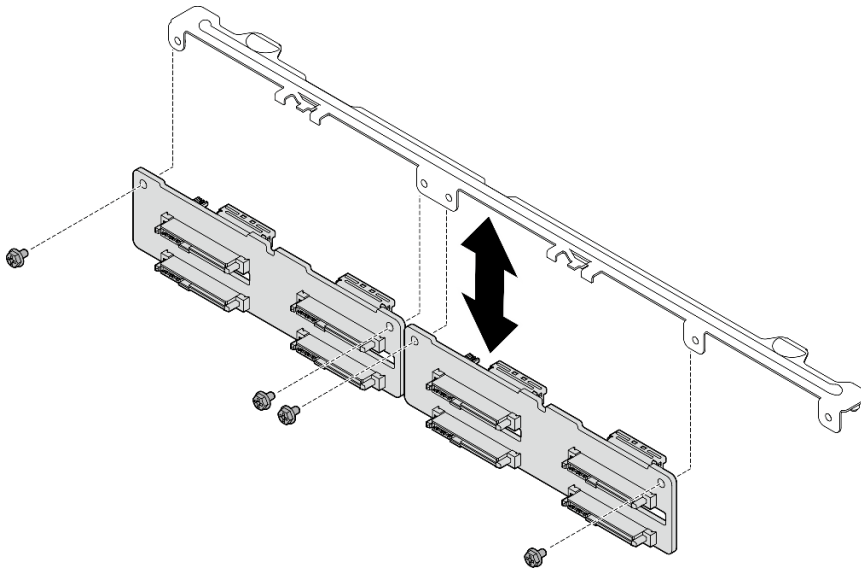
圖例 39. 卸下前方 2.5 吋硬碟背板
