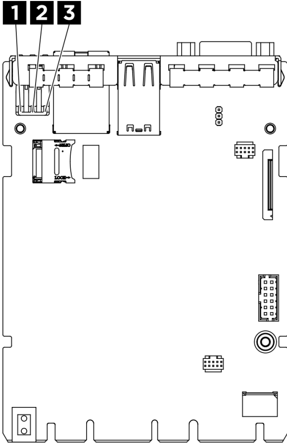
圖例 430. 系統 I/O 板上的 LED
