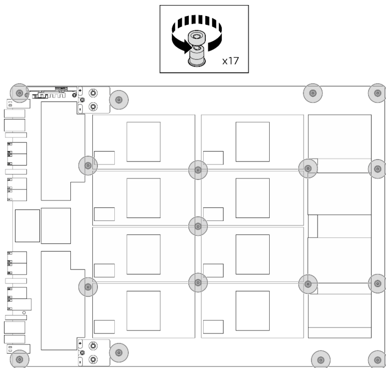
圖例 117. 卸下螺絲
