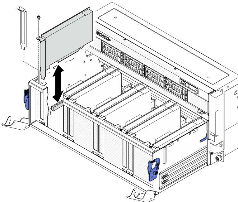
圖例 312. 卸下正面 PCIe 配接卡
