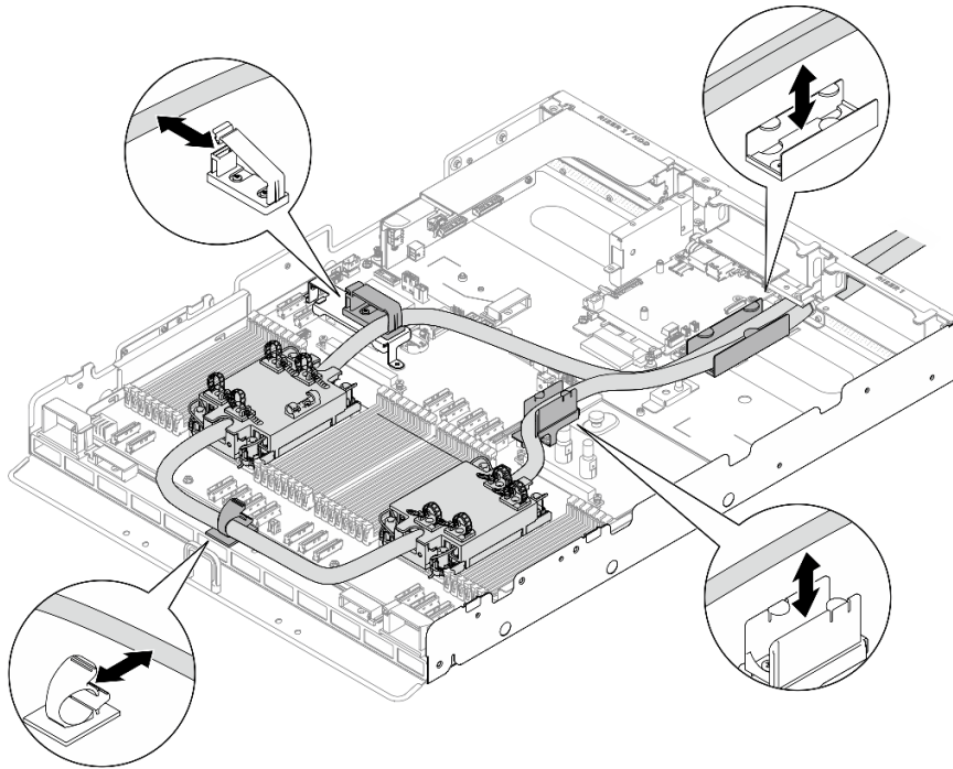
圖例 289. 安裝軟管和模組
