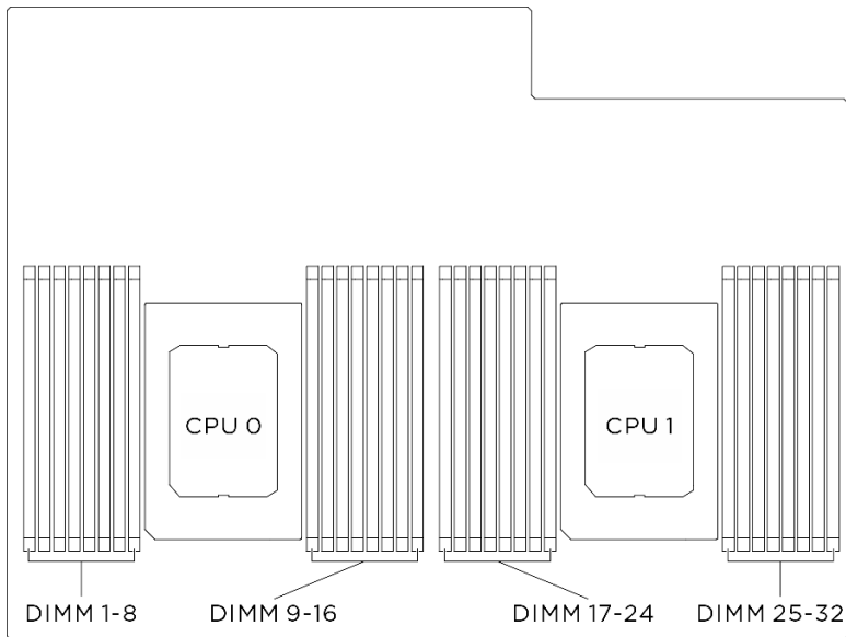
圖例 306. 記憶體模組和處理器佈置
