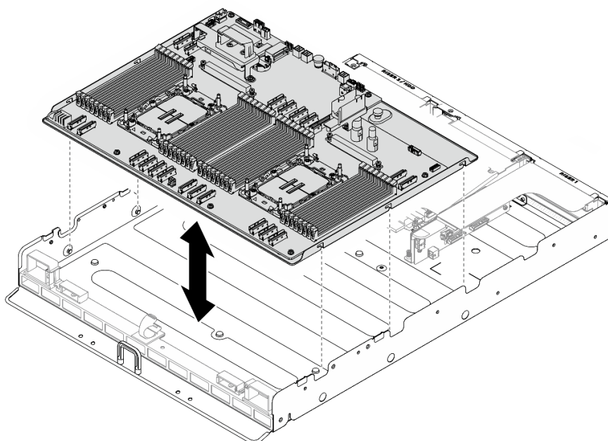
圖例 438. 卸下主機板
