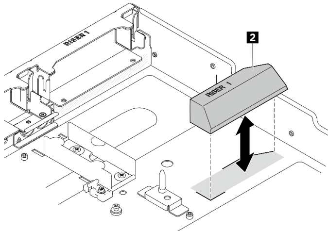
圖例 52. 從機箱卸下 DPU 空氣擋板
