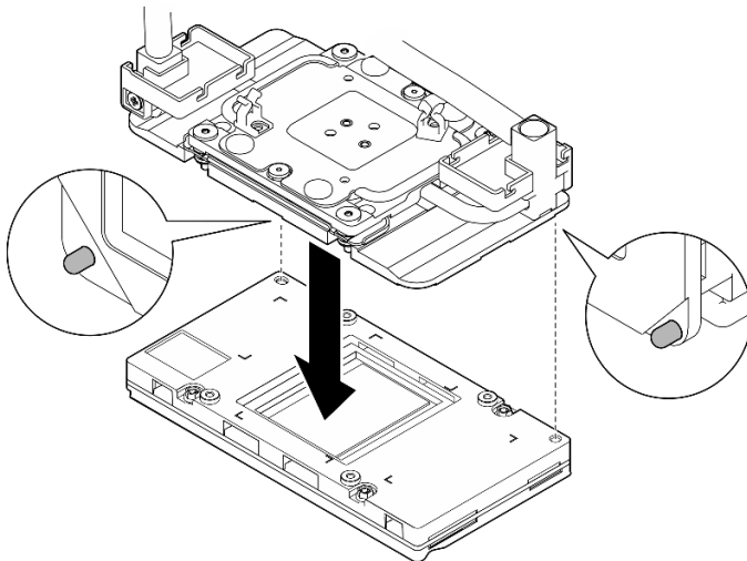
圖例 203. 調整 GPU 水冷板
