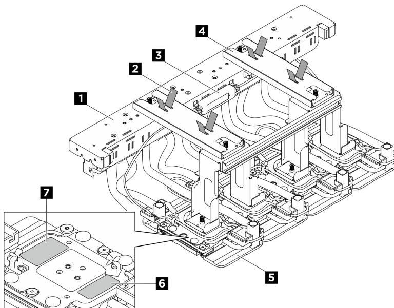
圖例 187. 後方 H100/H200 GPU 水冷板模組元件識別
