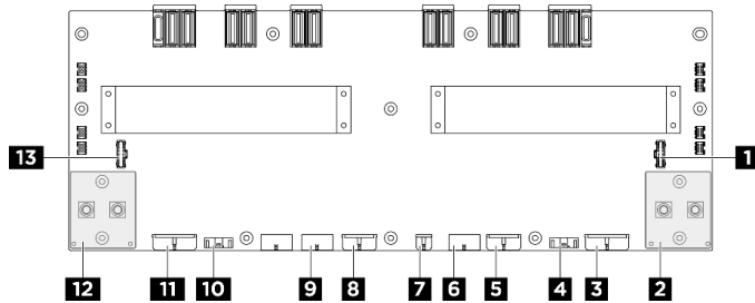
圖例 397. 電源配送板接頭
