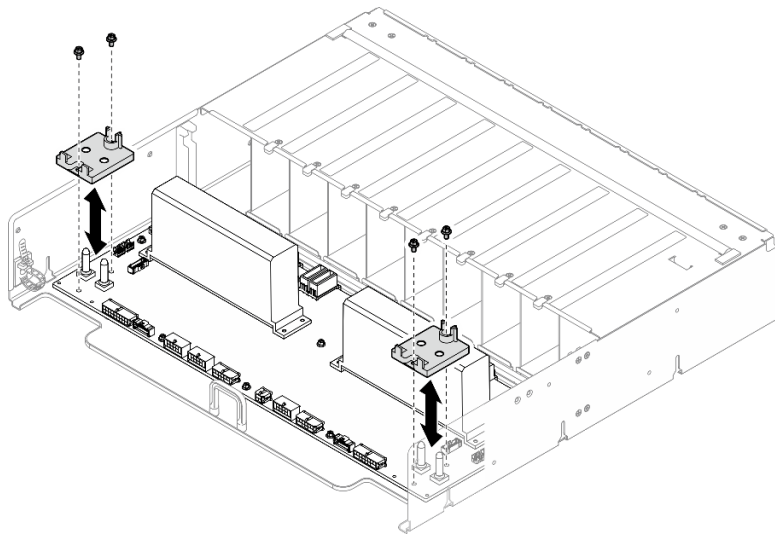
圖例 348. 安裝纜線固定器
