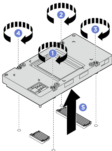
圖例 248. 卸下 GPU
