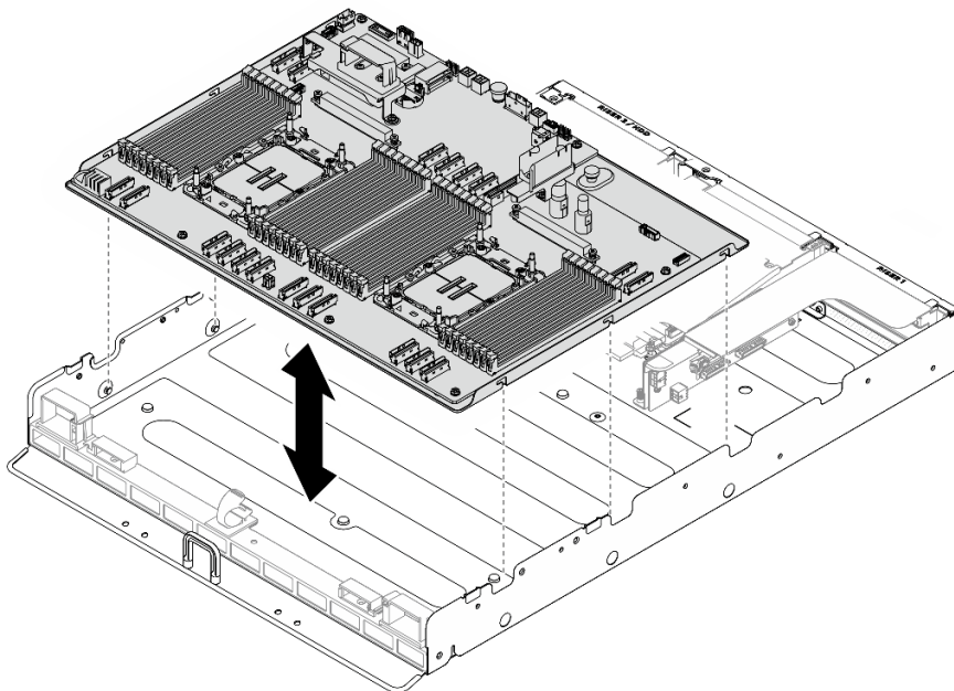
圖例 384. 卸下主機板
