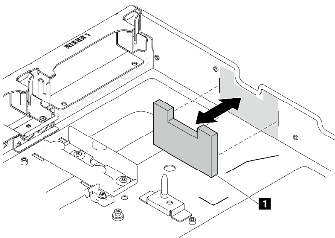
圖例 61. 將擴充卡插槽 1 DPU 空氣擋板安裝到機箱
