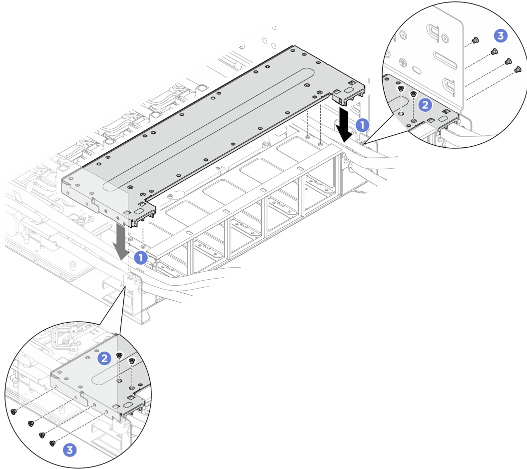
圖例 91. 安裝後方風扇機盒支撐托架
