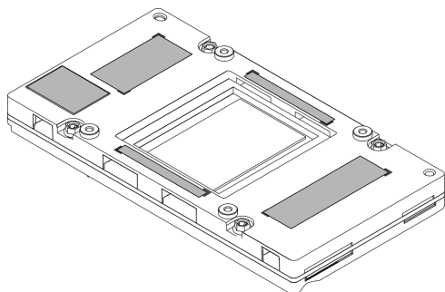
圖例 222. 清除 GPU 上的 PCM 和油灰墊
