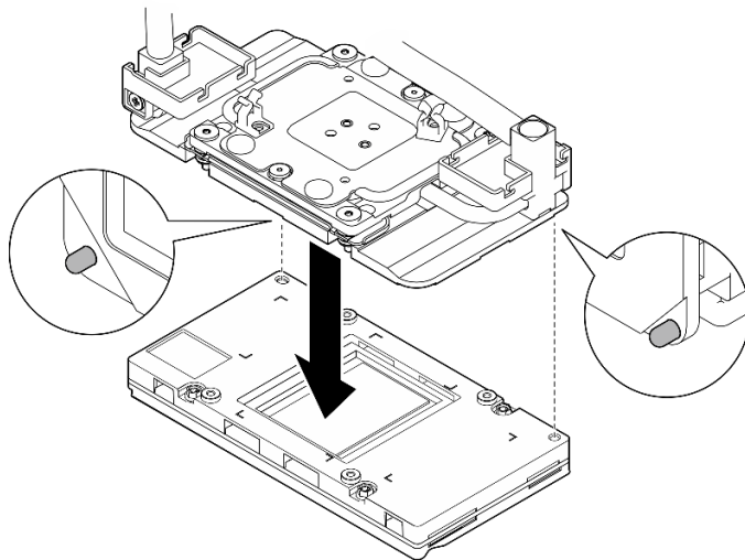
圖例 177. 調整 GPU 水冷板
