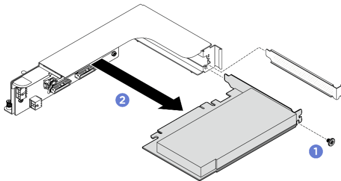
圖例 322. 卸下背面 PCIe 配接卡
