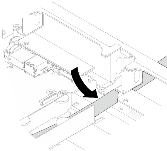
圖例 290. 安裝軟管
