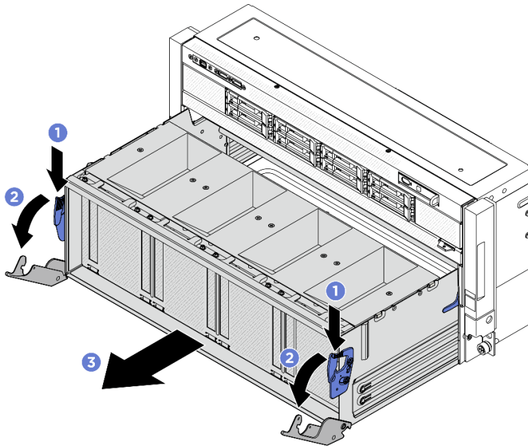
圖例 98. 將 PCIe 交換器滑動箱從停止位置卸下
