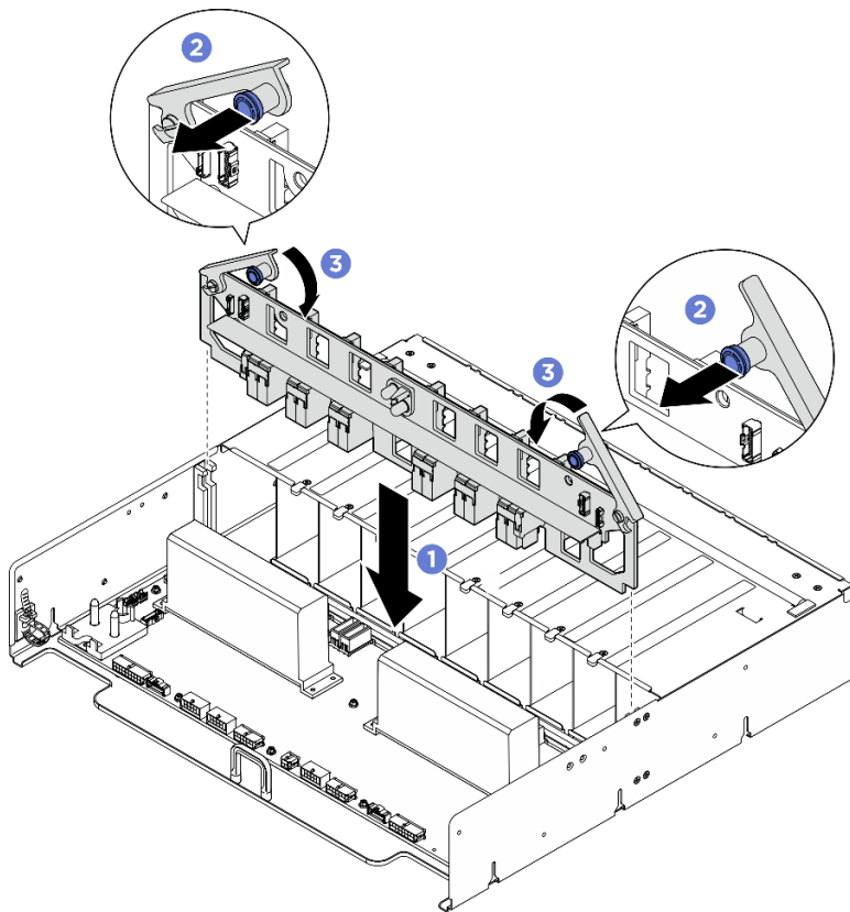
圖例 366. 安裝 PSU 轉插卡
