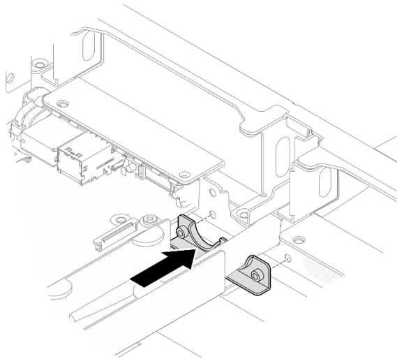
圖例 291. 安裝水管固定器
