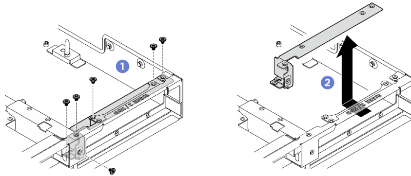
圖例 369. 卸下背面框架支撐托架
