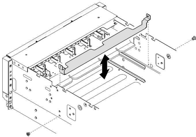
圖例 99. 卸下 GPU 接頭保護托架
