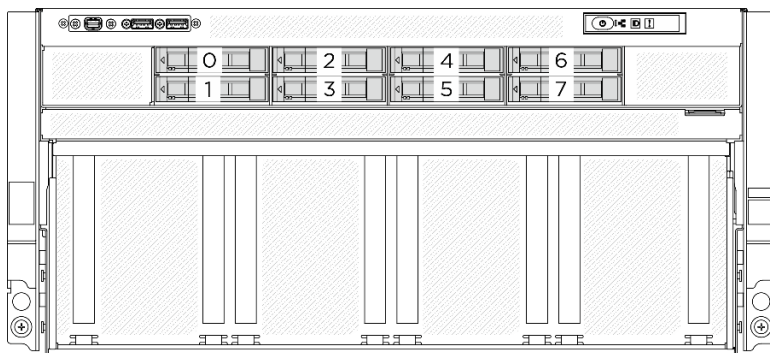
圖例 29. 前方 2.5 吋機槽編號
