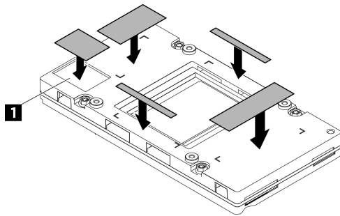
圖例 253. 更換 GPU 油灰墊
