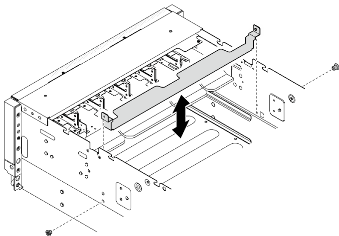
圖例 116. 卸下 GPU 接頭保護托架
