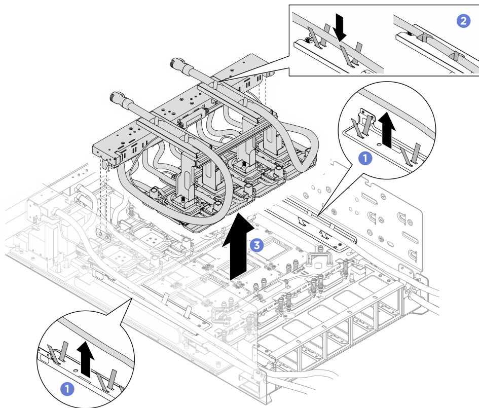
圖例 194. 卸下後方 H100/H200 GPU 水冷板模組
