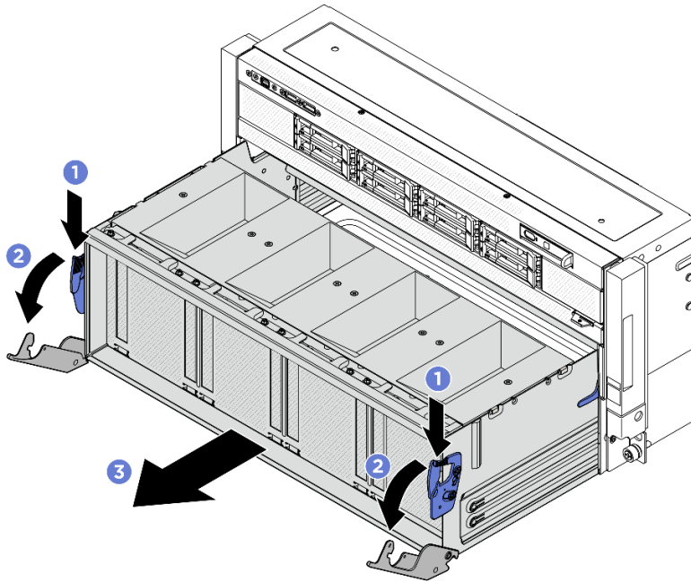
圖例 334. 將 PCIe 交換器滑動箱從停止位置卸下
