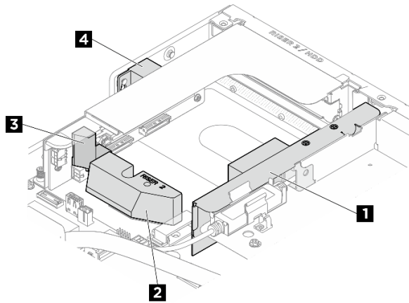
圖例 64. DPU 空氣擋板在擴充卡 2 插槽中的位置
