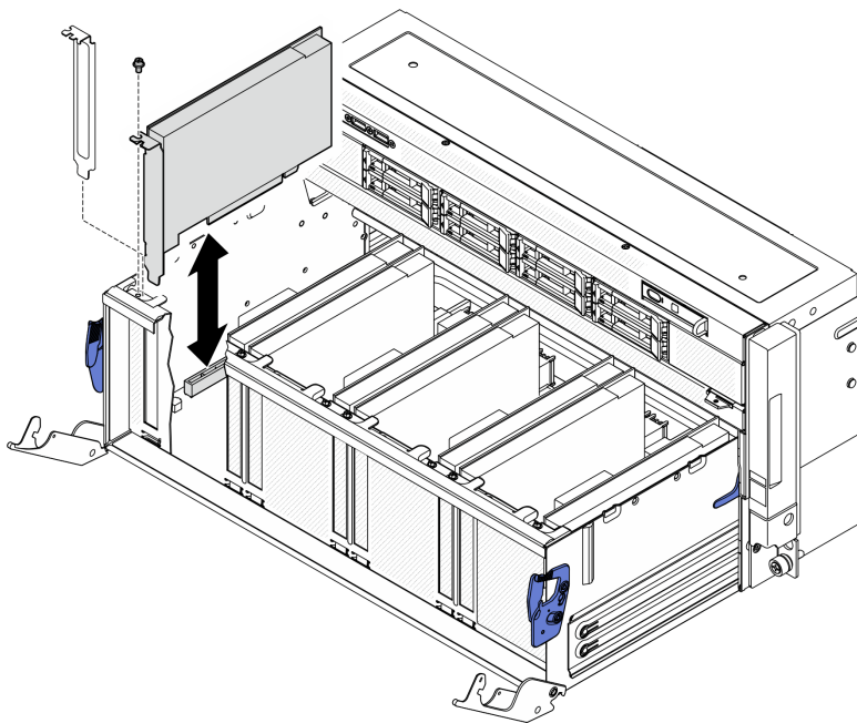
圖例 313. 安裝正面 PCIe 配接卡
