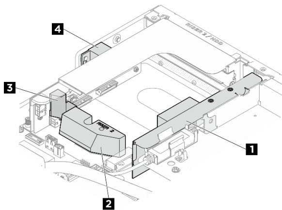
圖例 54. DPU 空氣擋板在擴充卡 2 插槽中的位置
