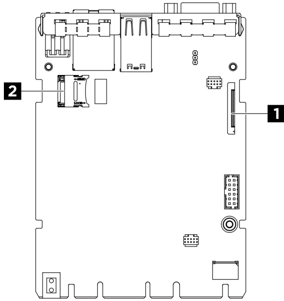
圖例 17. 系統 I/O 板接頭
