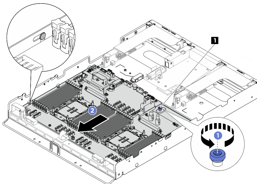
圖例 437. 鬆開主機板
