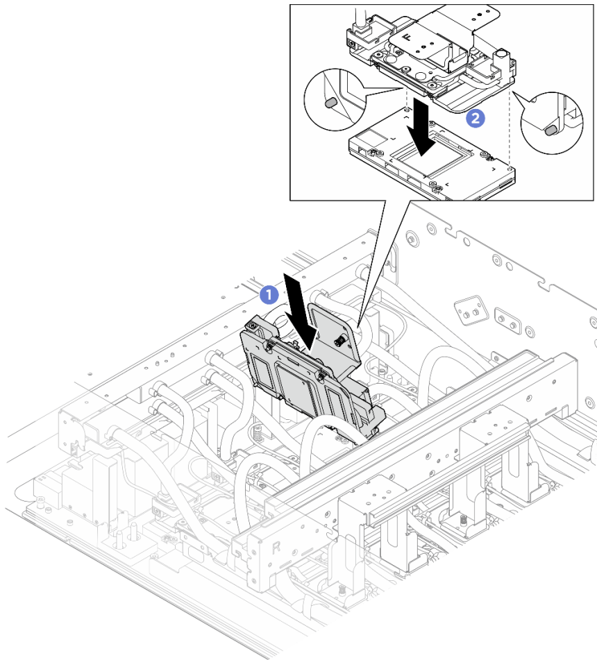
圖例 231. 放置 GPU 水冷板
