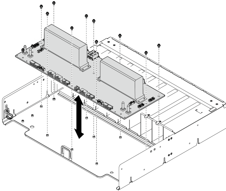
圖例 360. 卸下電源配送板
