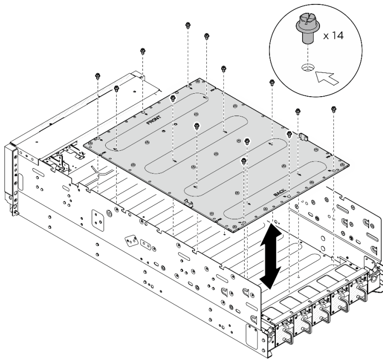
圖例 131. 安裝 GPU 複合體配接器板
