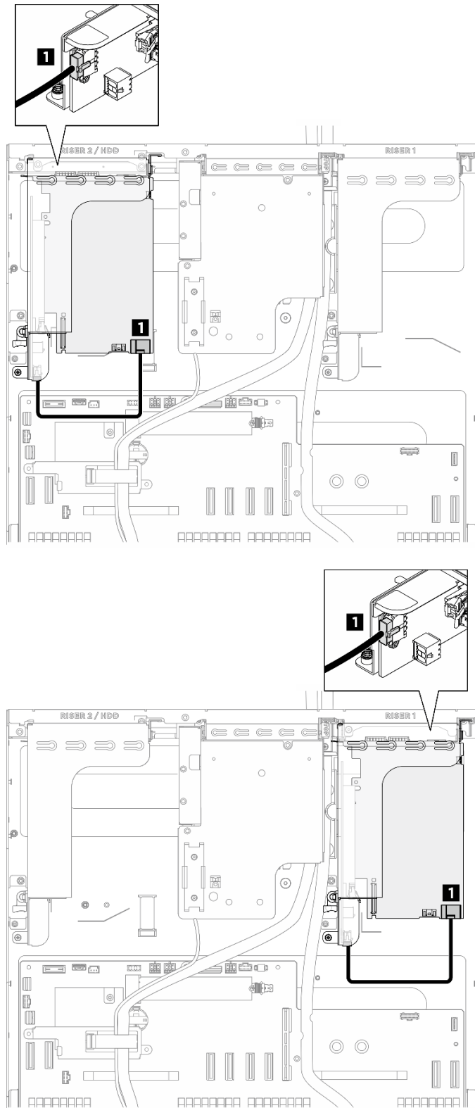
圖例 417. DPU 電源線佈線
