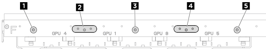
圖例 221. 維修托架和 GPU 水冷板組件安裝位置
