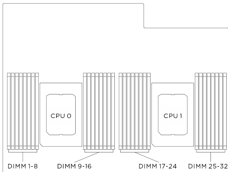
圖例 304. 記憶體模組和處理器佈置
