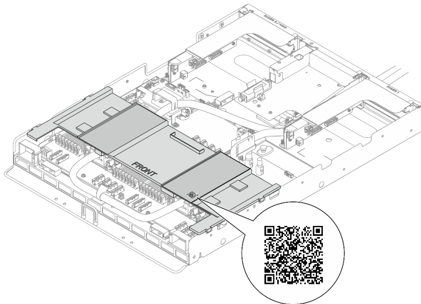
圖例 21. 服務標籤和 QR 代碼
