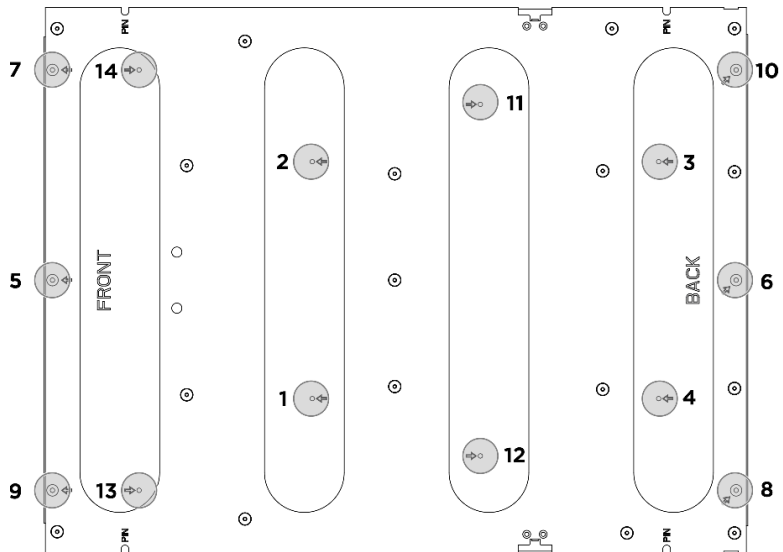
圖例 130. GPU 複合體配接器板螺絲順序
