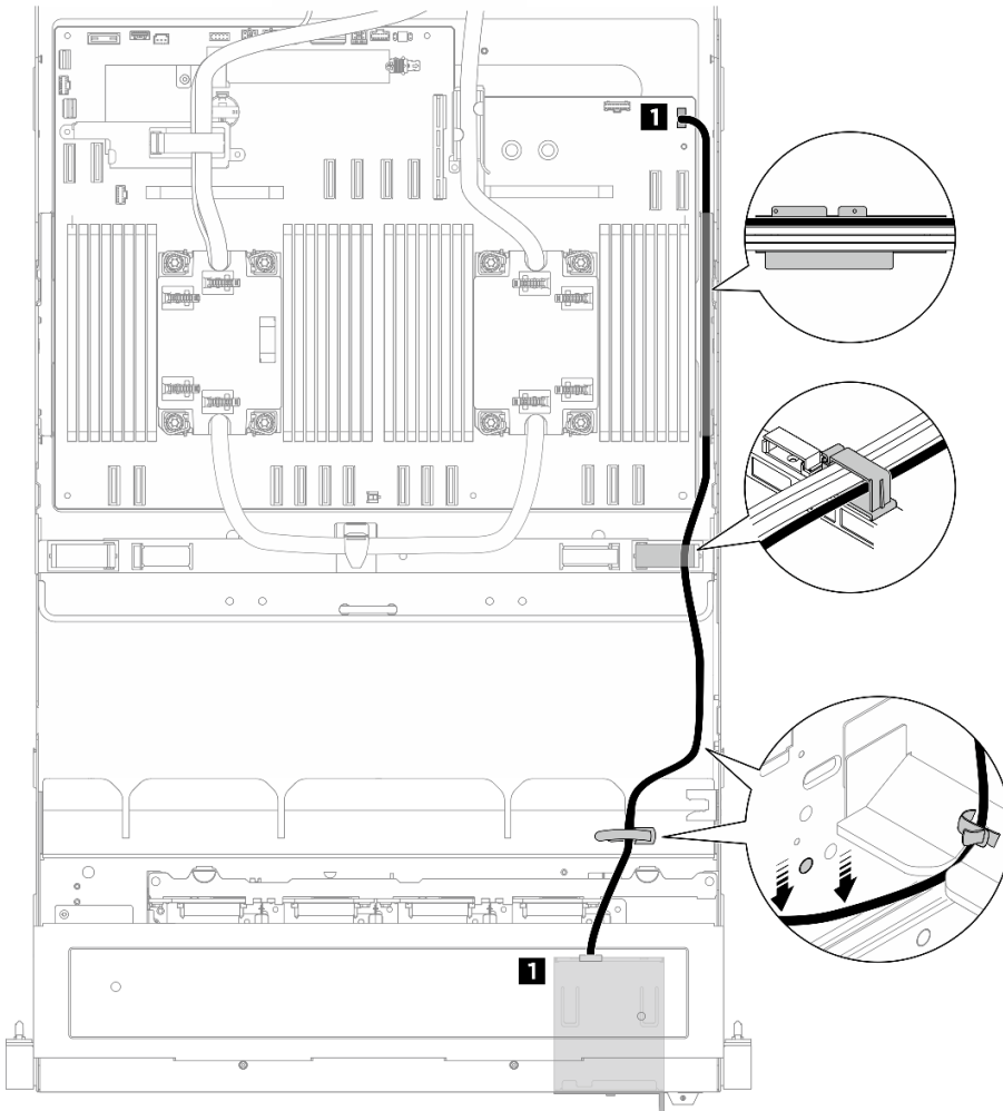
圖例 408. 整合式診斷面板纜線佈線
