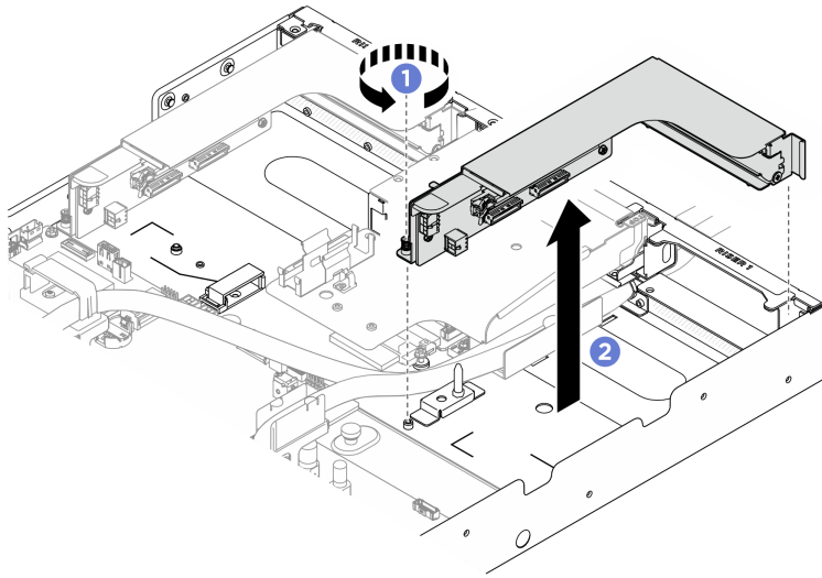
圖例 319. 卸下插槽 1 中的 PCIe 擴充卡組件
