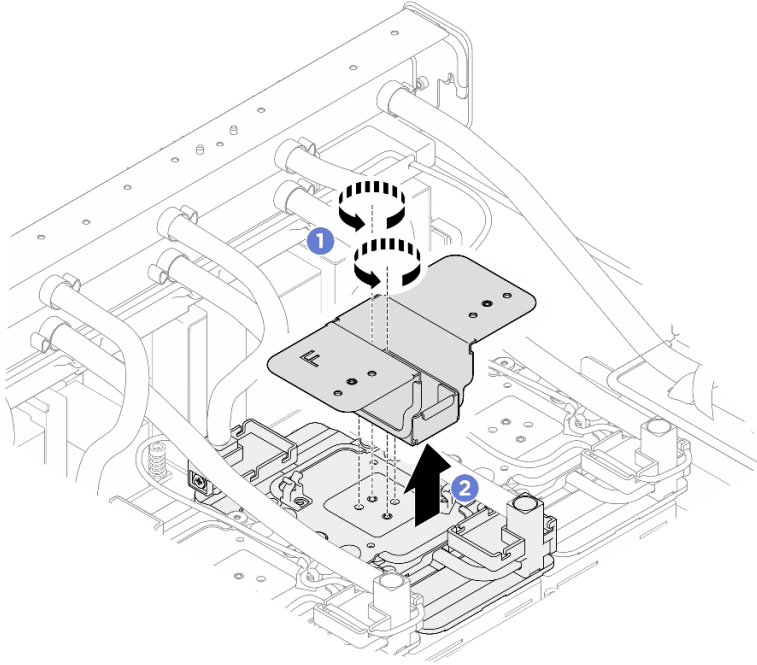
圖例 232. 卸下維修托架
