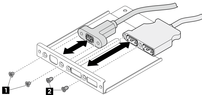
圖例 93. 卸下正面 I/O 模組纜線
