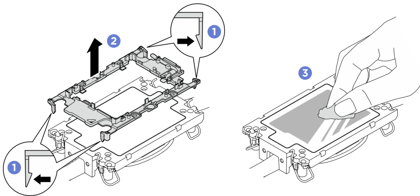
圖例 281. 將處理器支架與水冷板分開
