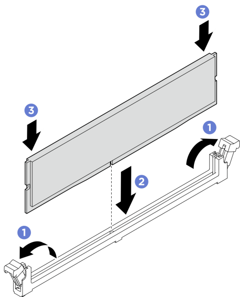
圖例 307. 安裝記憶體模組
