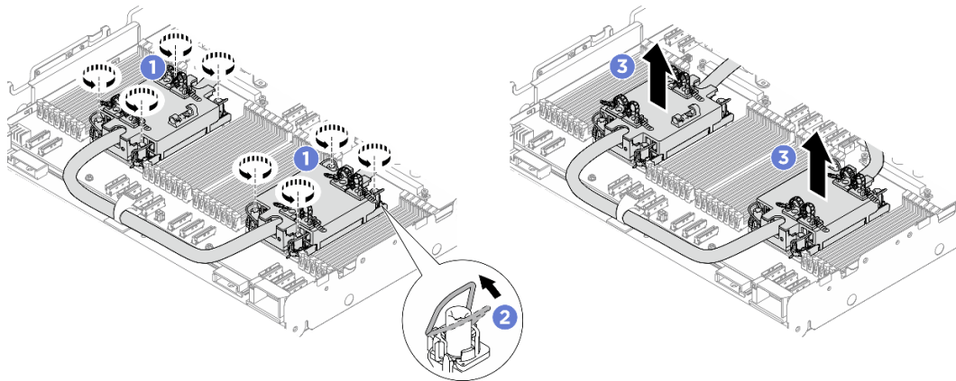
圖例 279. 卸下 DWCM
