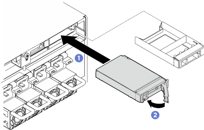
圖例 36. 安裝背面 2.5 吋熱抽換硬碟
