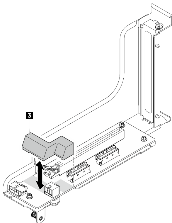
圖例 63. 將 DPU 空氣擋板安裝到 PCIe 擴充卡
