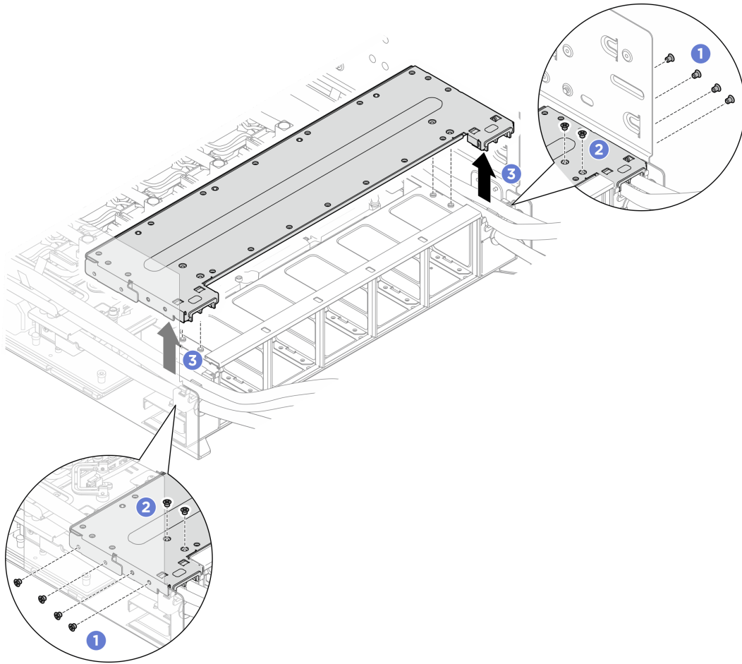
圖例 159. 卸下後方風扇機盒支撐托架
