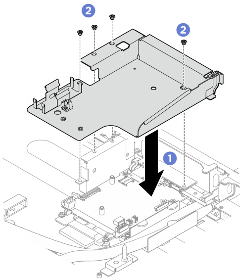
圖例 295. 安裝洩漏感應器模組匣托架
