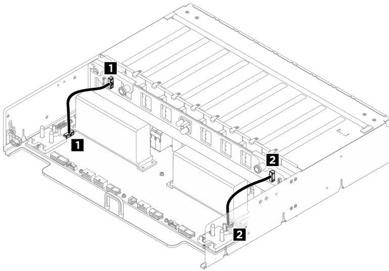
圖例 414. PSU 轉插卡到電源配送板纜線佈線
