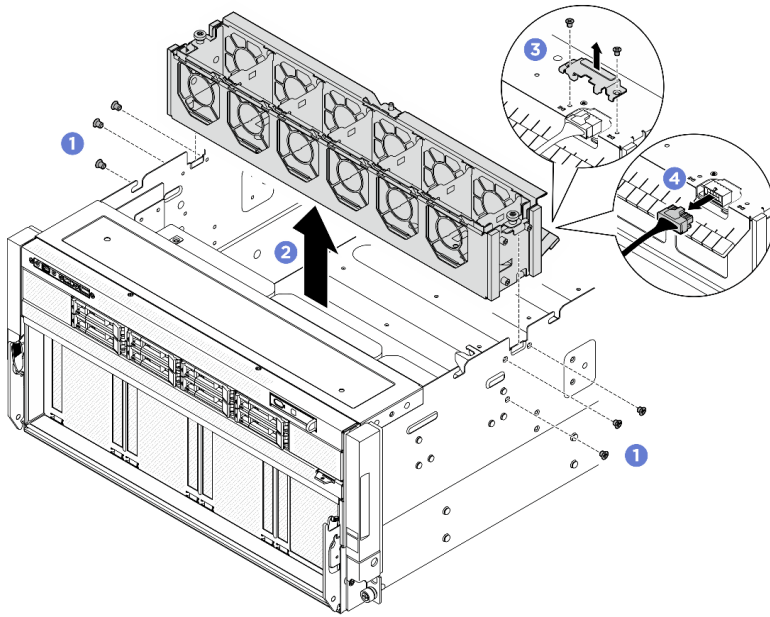
圖例 72. 卸下風扇機盒
