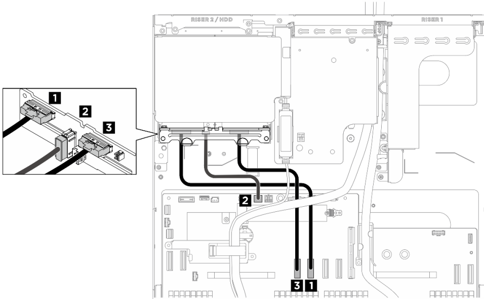
圖例 402. 後方 2.5 吋硬碟背板纜線佈線
