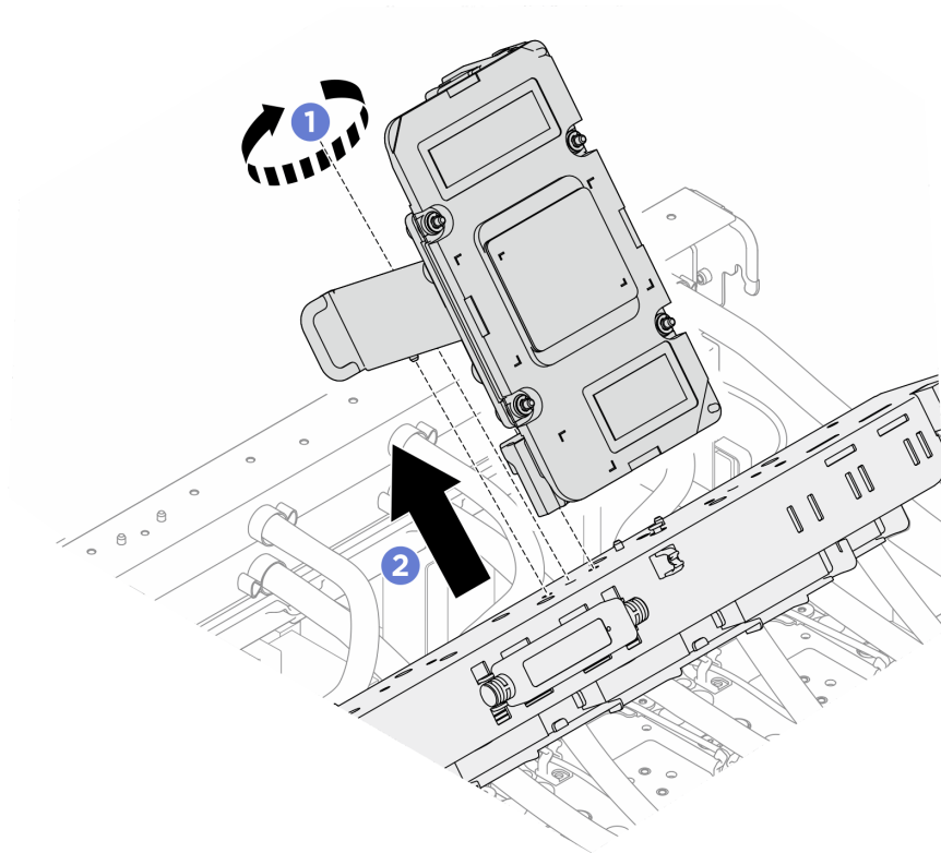
圖例 254. 卸下維修托架和 GPU 水冷板組件
