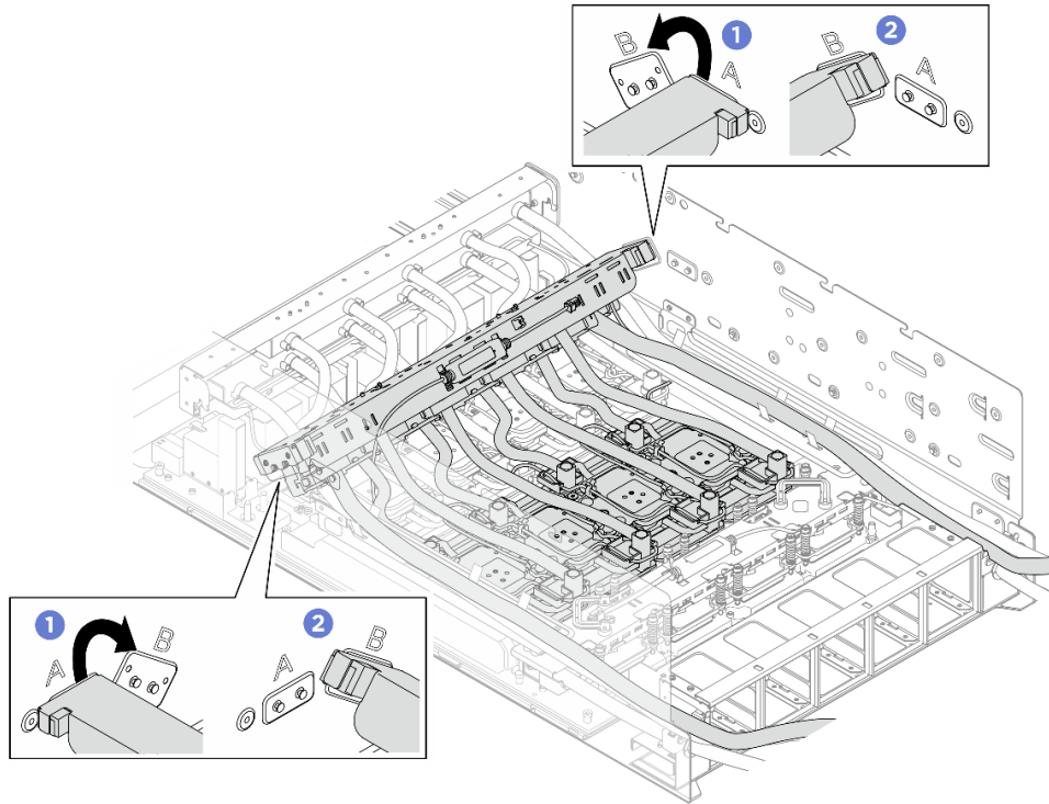
圖例 209. 重新放置後方 H100/H200 GPU 水冷板模組歧管
