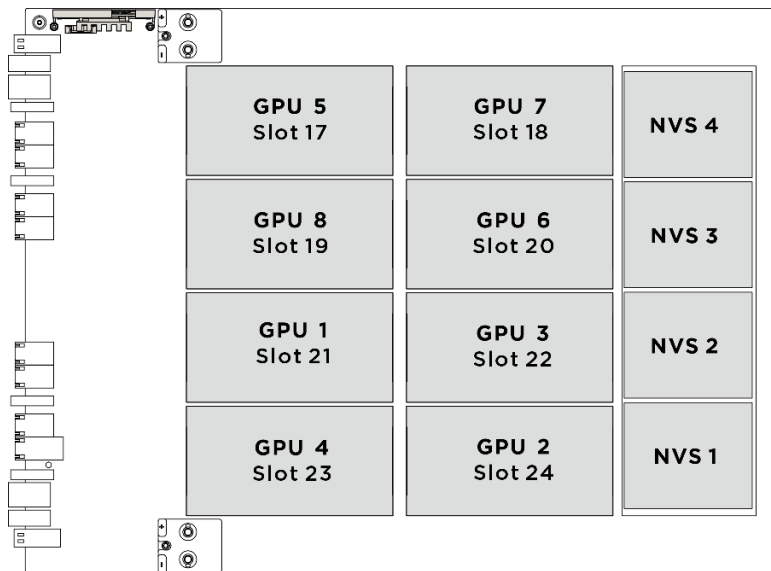
圖例 169. GPU 編號
