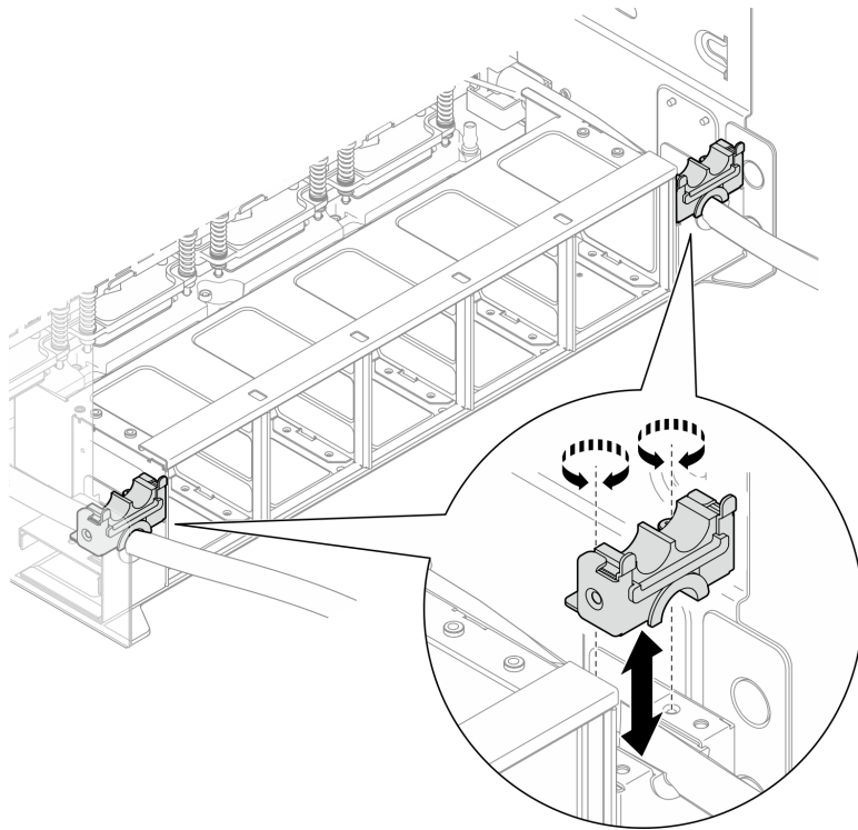
圖例 152. 安裝水管固定器 B/C
