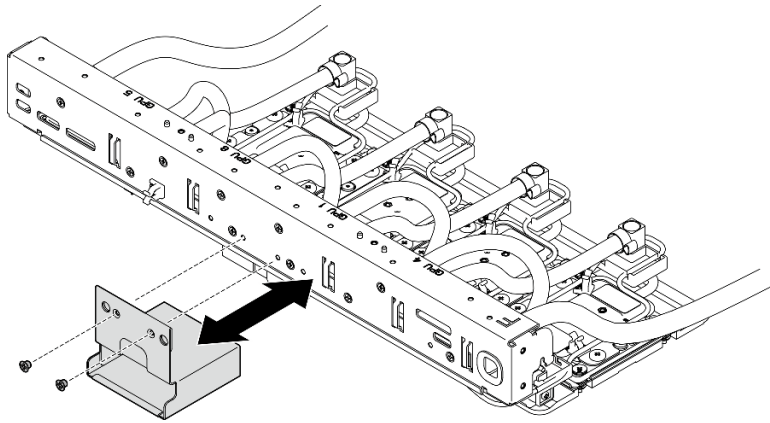
圖例 168. 卸下 GPU 纜線固定器
