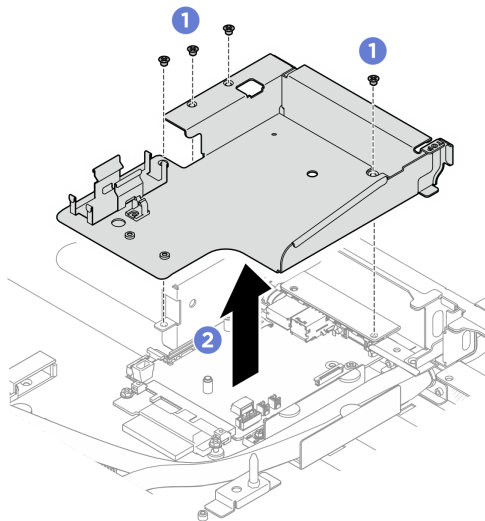
圖例 272. 卸下洩漏感應器模組匣托架
