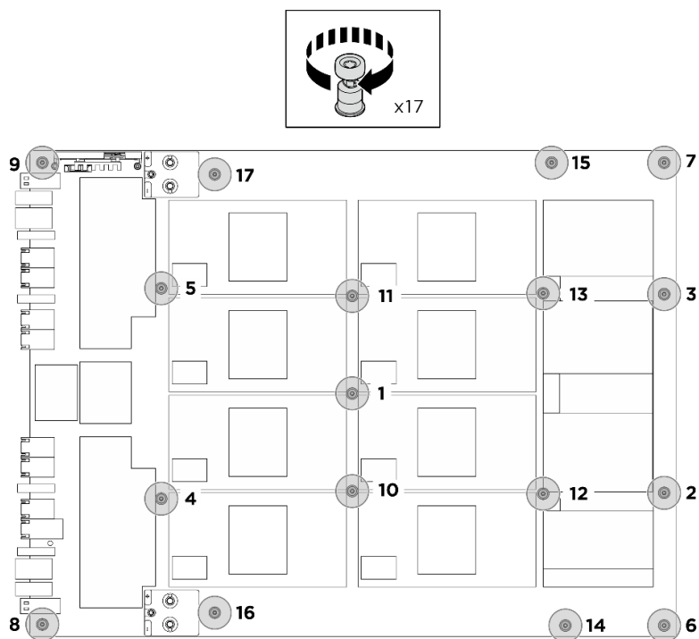
圖例 125. 安裝螺絲
