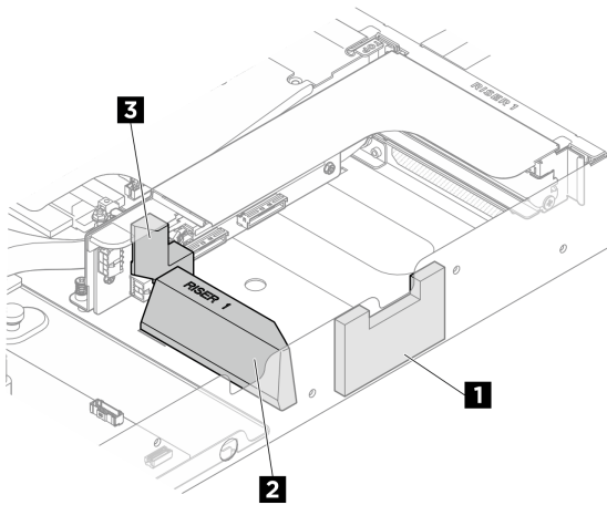
圖例 59. DPU 空氣擋板在擴充卡 1 插槽中的位置
