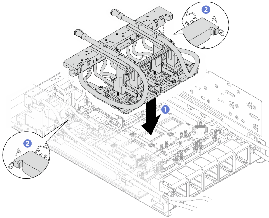
圖例 201. 安裝後方 H100/H200 GPU 水冷板模組
