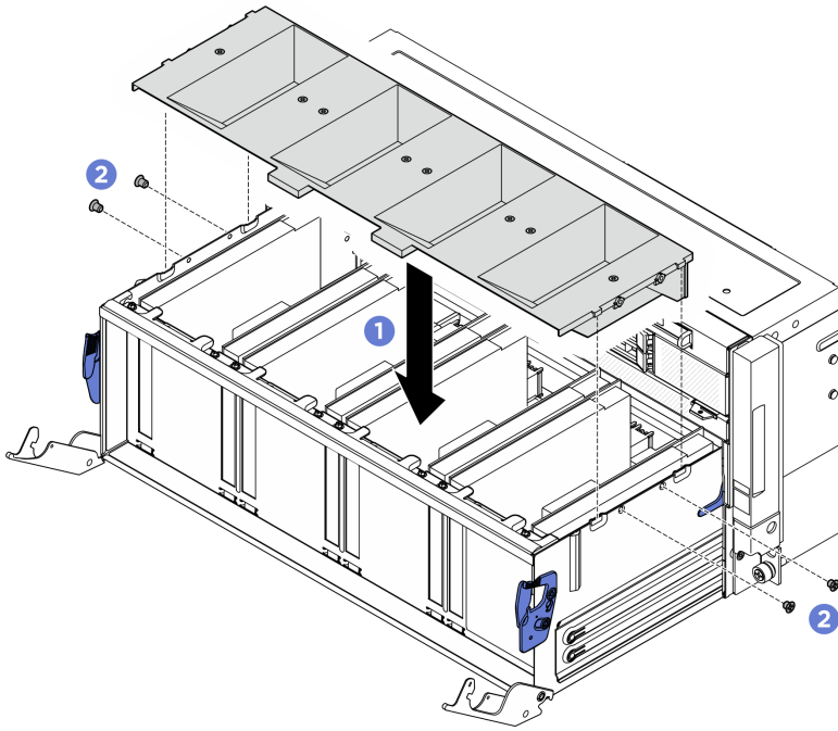
圖例 339. 安裝空氣擋板
