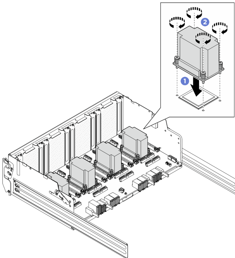
圖例 333. 安裝 PCIe 交換器板散熱槽
