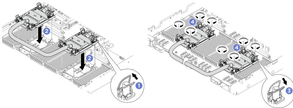
圖例 286. 安裝處理器連接 DWCM
