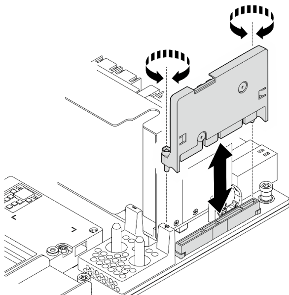
圖例 261. 安裝 HMC 卡
