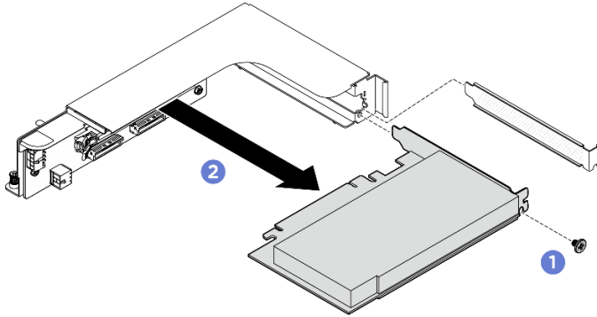
圖例 316. 卸下背面 PCIe 配接卡
