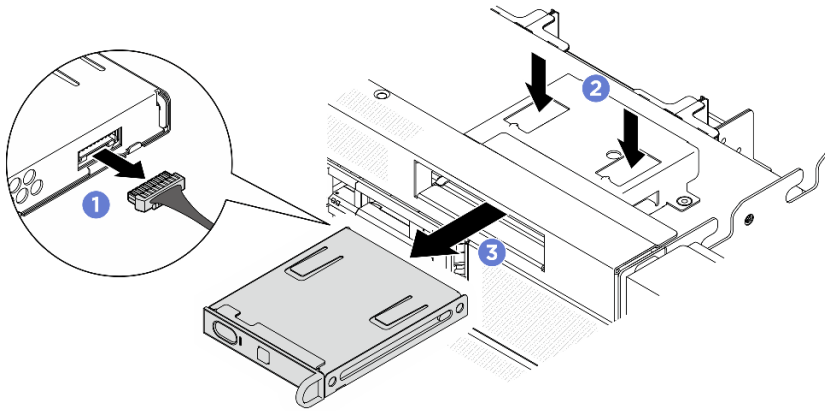
圖例 262. 卸下整合式診斷面板
