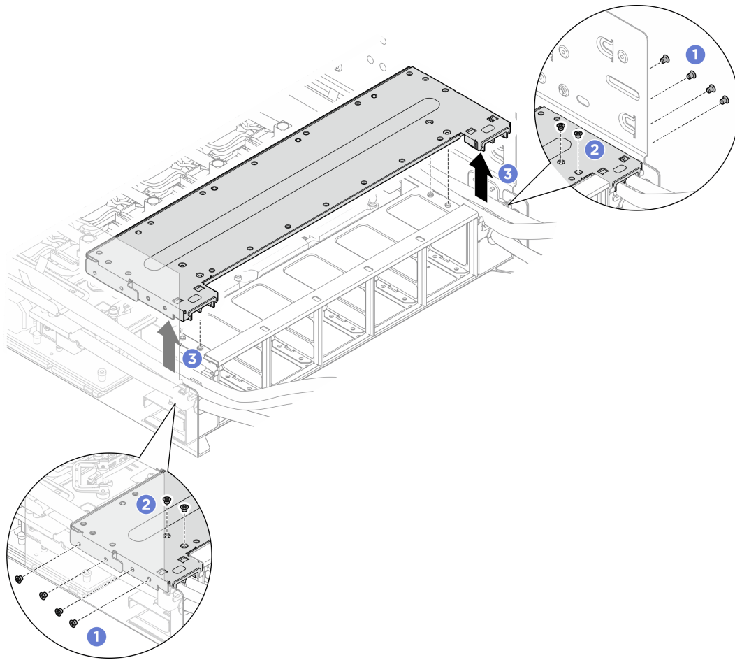
圖例 136. 卸下後方風扇機盒支撐托架
