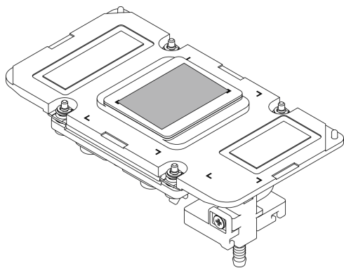
圖例 223. 擦掉水冷板上的 PCM 和油灰墊
