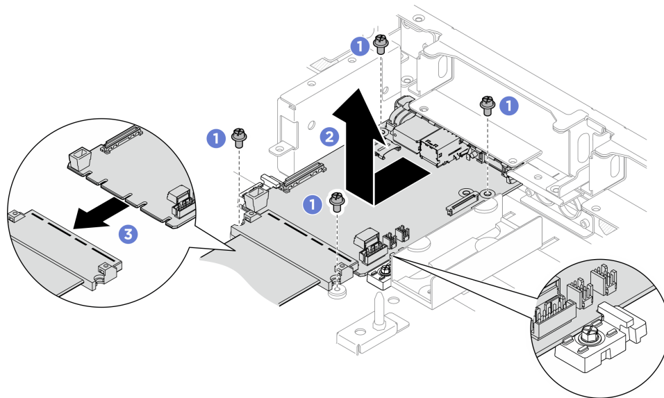
圖例 380. 卸下系統 I/O 板
