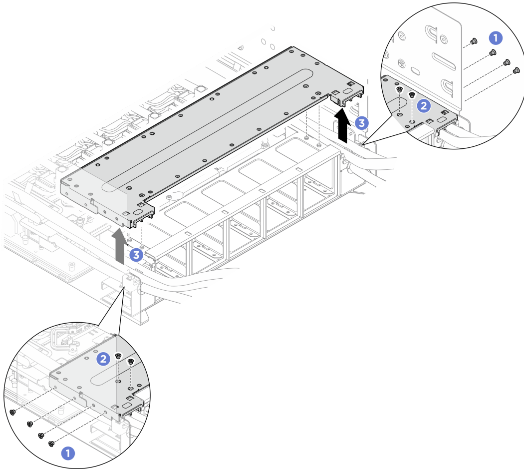
圖例 189. 卸下後方風扇機盒支撐托架
