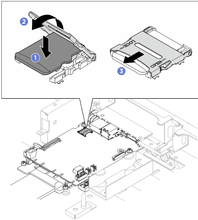
圖例 309. 安裝 MicroSD 卡
