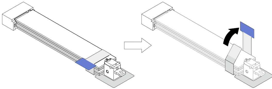
圖例 298. 卸下 M.2 卡板固定器
