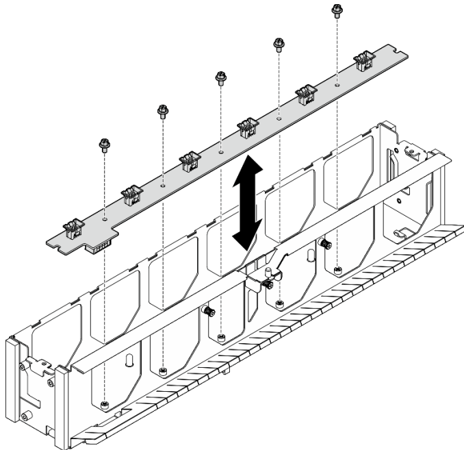
圖例 83. 卸下前方風扇控制板
