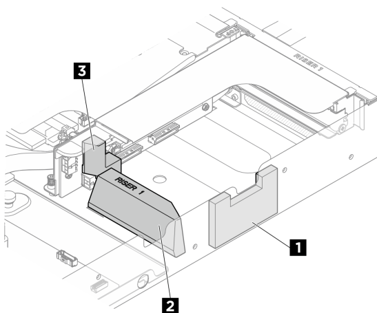
圖例 50. DPU 空氣擋板在擴充卡 1 插槽中的位置
