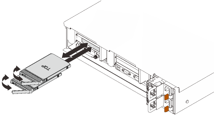
그림 53. 7mm 드라이브 제거
