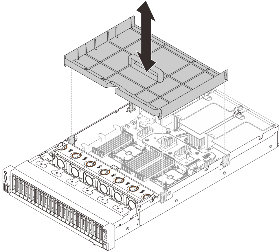
그림 71. 시스템 공기 조절 장치 제거
