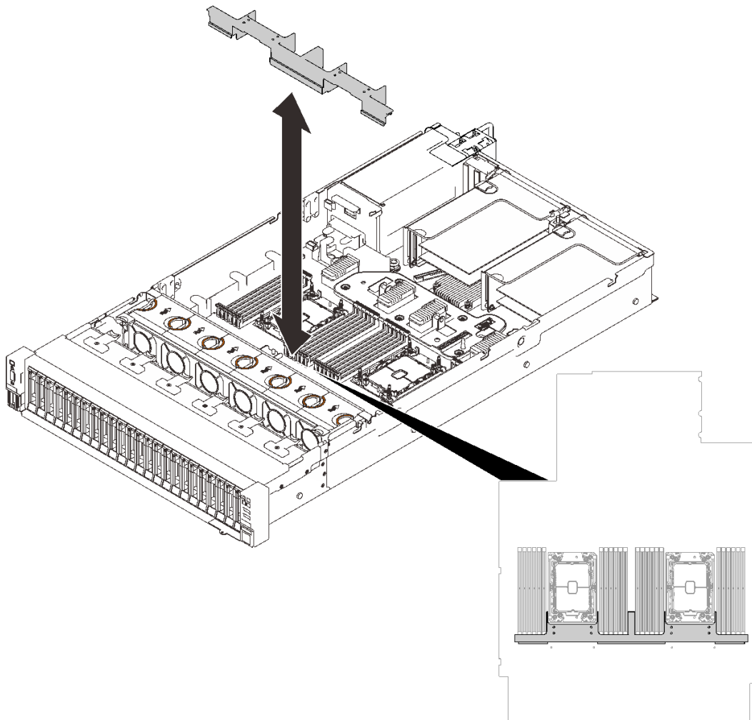
그림 83. 확장 트레이 공기 조절 장치 설치
