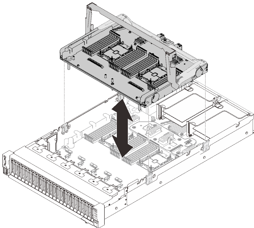
그림 74. 프로세서 및 메모리 확장 트레이 제거
