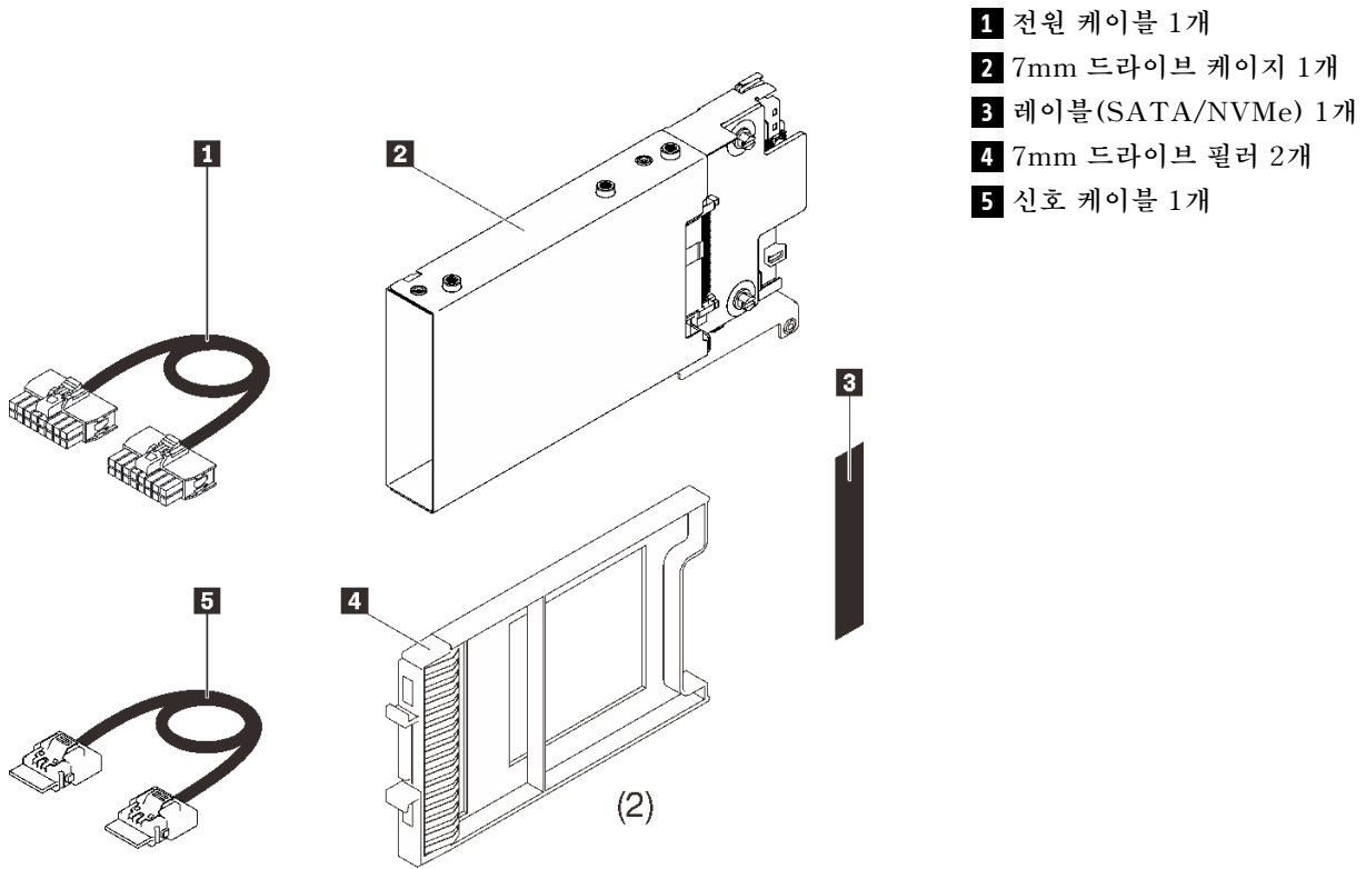
그림 34. 7mm 드라이브 케이지 키트
