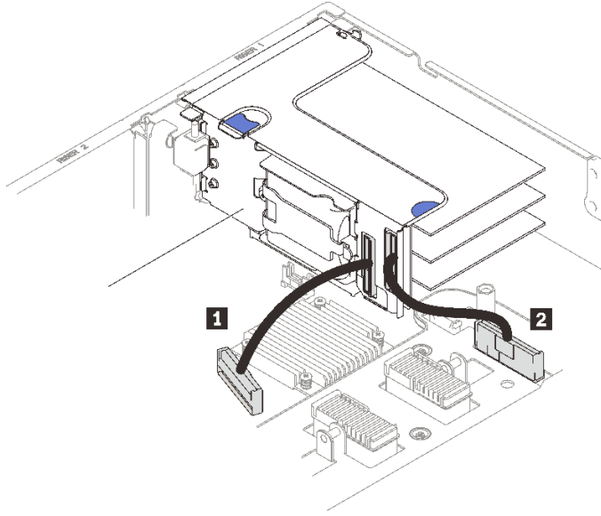
그림 69. x16/x16/x16 라이저의 PCIe 케이블을 시스템 보드에 연결
