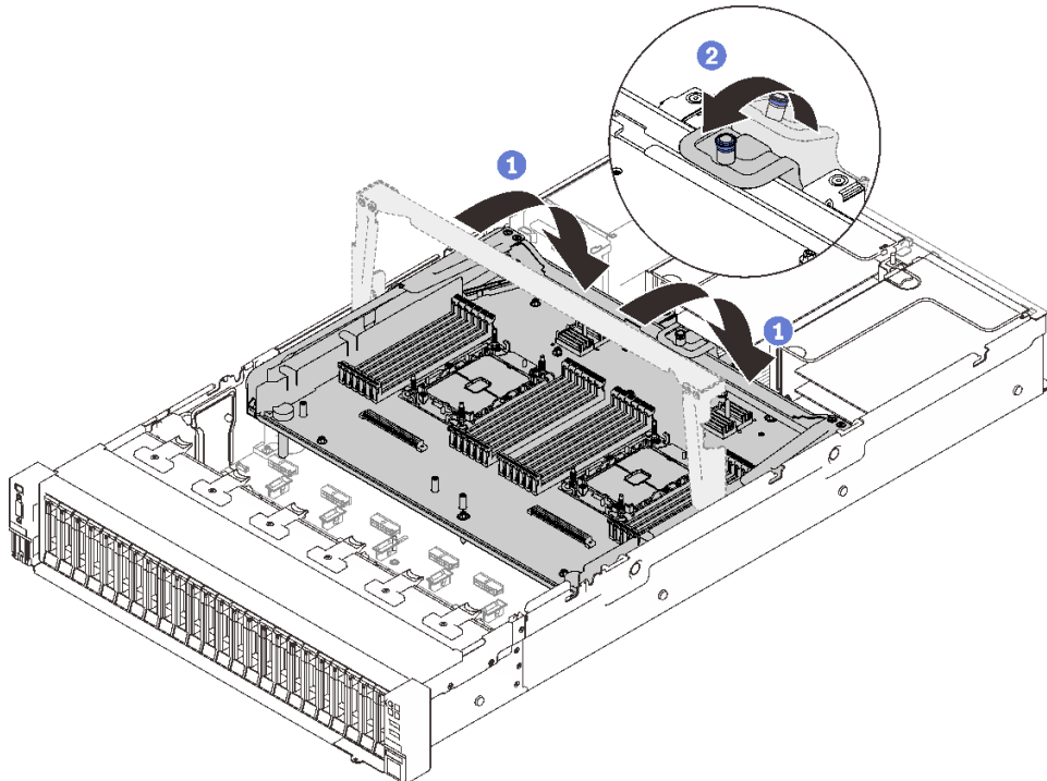
그림 86. 프로세서 및 메모리 확장 트레이 고정
