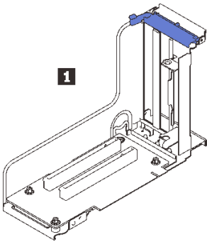
그림 37. x16/x16 (x8 레인) FH/HL PCIe 라이저 카드
