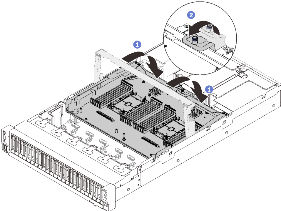
그림 24. 프로세서 및 메모리 확장 트레이 고정
