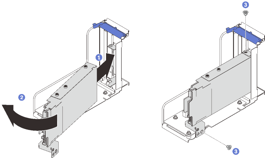
그림 82. 라이저에 7mm 드라이브 케이스를 설치하십시오.
