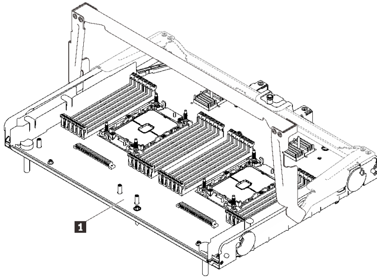
그림 43. 프로세서 및 메모리 확장 트레이
