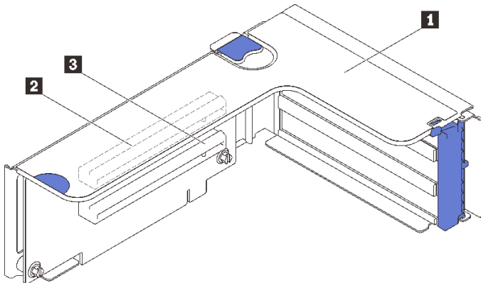
그림 36. x16/x16(x8 레인) PCIe 라이저 카드 커넥터
