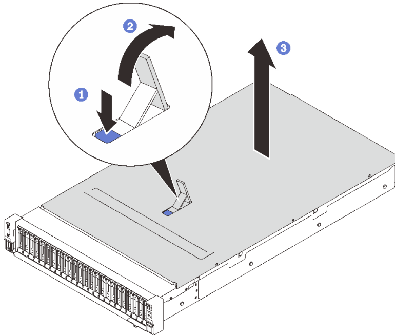
그림 52. 윗면 덮개 제거
