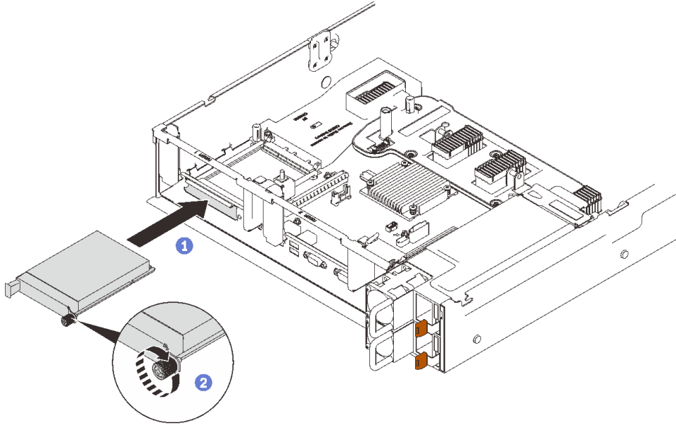
그림 67. OCP 이더넷 어댑터 설치
