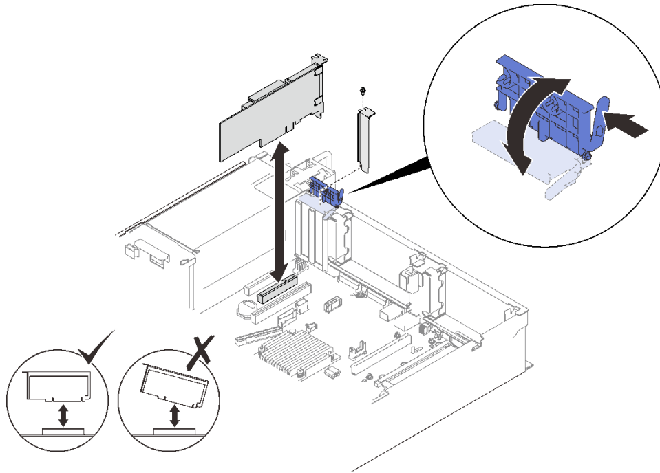
그림 59. 시스템 보드에 어댑터 설치
