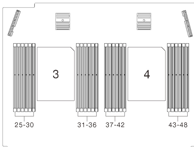
그림 77. 프로세서 및 메모리 확장 트레이의 프로세서 3 및 4 위치
