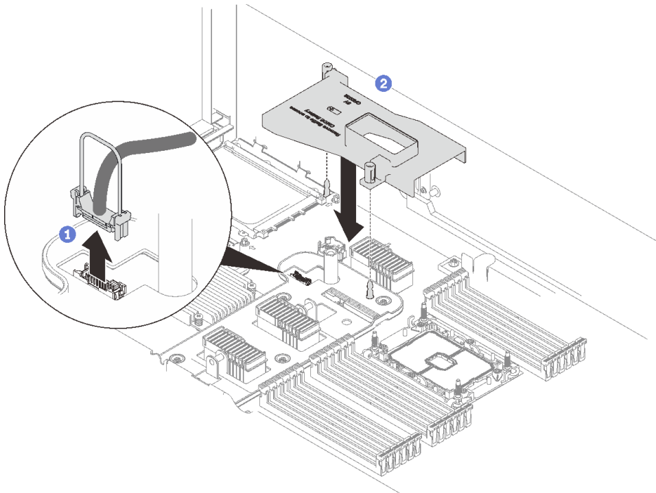
그림 66. OCP 어댑터 공기 조절 장치 설치 중
