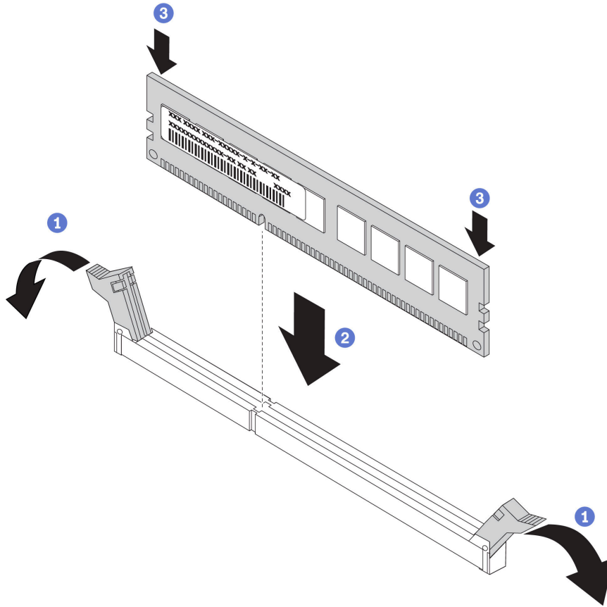
그림 80. 메모리 모듈 설치
