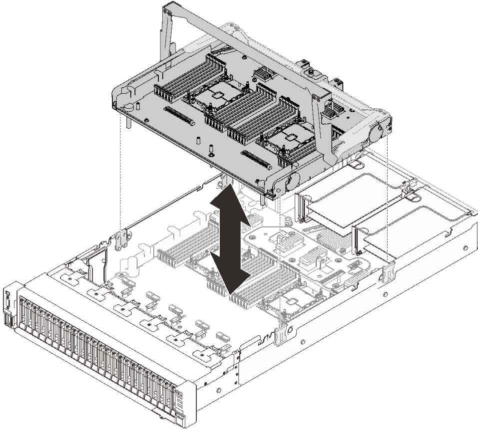
그림 22. 프로세서 및 메모리 확장 트레이 설치
