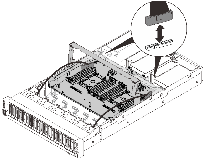
그림 85. 확장 트레이에 케이블 연결
