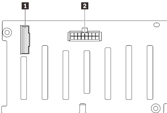
그림 28. SAS/SATA 드라이브 백플레인 커넥터
