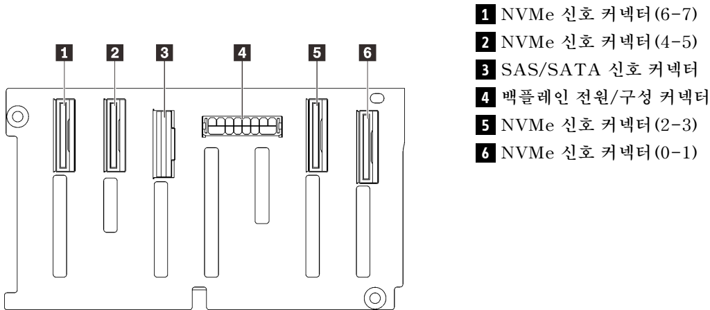
그림 30. AnyBay/NVMe 드라이브 백플레인 커넥터
