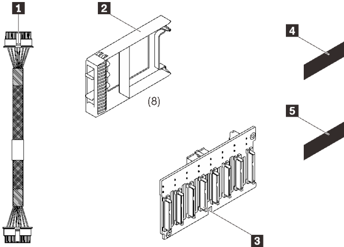
그림 27. 2.5인치 8베이 SAS/SATA 백플레인 키트
