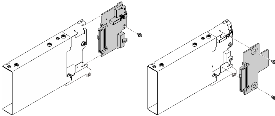
그림 81. 7mm 드라이브 백플레인 설치
