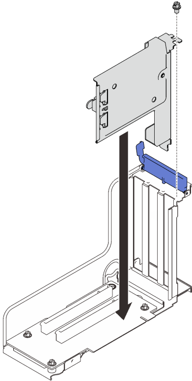
그림 64. 라이저에 플래시 전원 모듈 브래킷 설치 중
