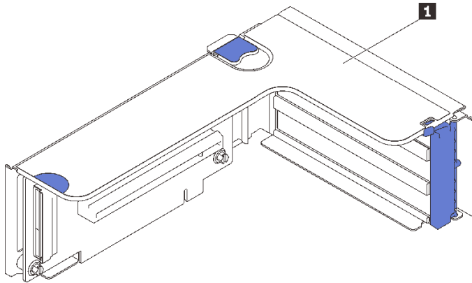
그림 41. x16/x16 FH/HL PCIe 라이저 키트
