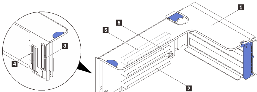
그림 40. x16/x16/x16 PCIe 라이저 카드 커넥터
