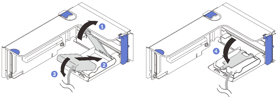
그림 65. 플래시 전원 모듈 설치
