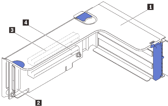
그림 42. x16/x16 PCIe 라이저 카드 커넥터
