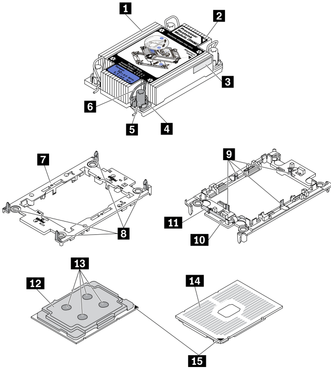
그림 78. PHM 구성 요소
