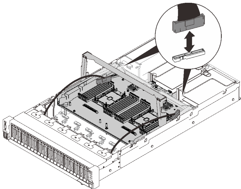
그림 73. PCIe 케이블 분리
