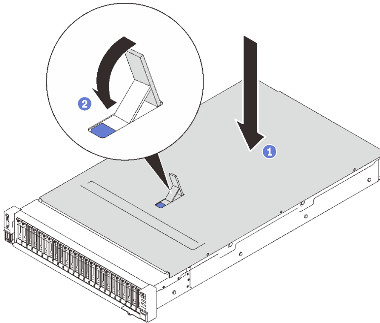
그림 88. 윗면 덮개 설치
