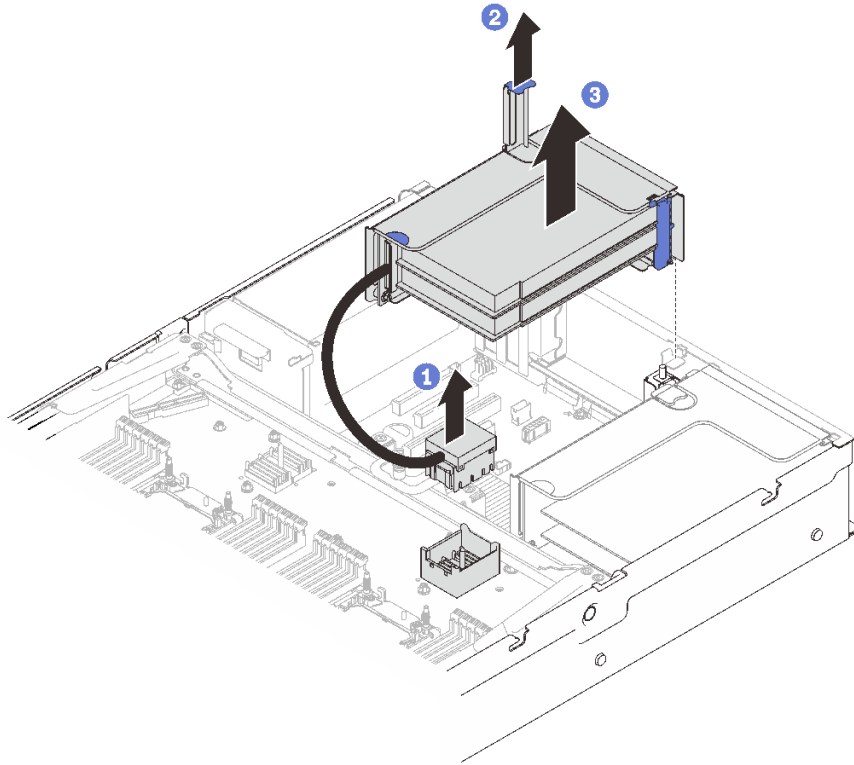
그림 58. 영역 2에서 PCIe 라이저 어셈블리 제거
