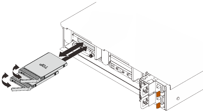
그림 46. 7mm 드라이브 설치
