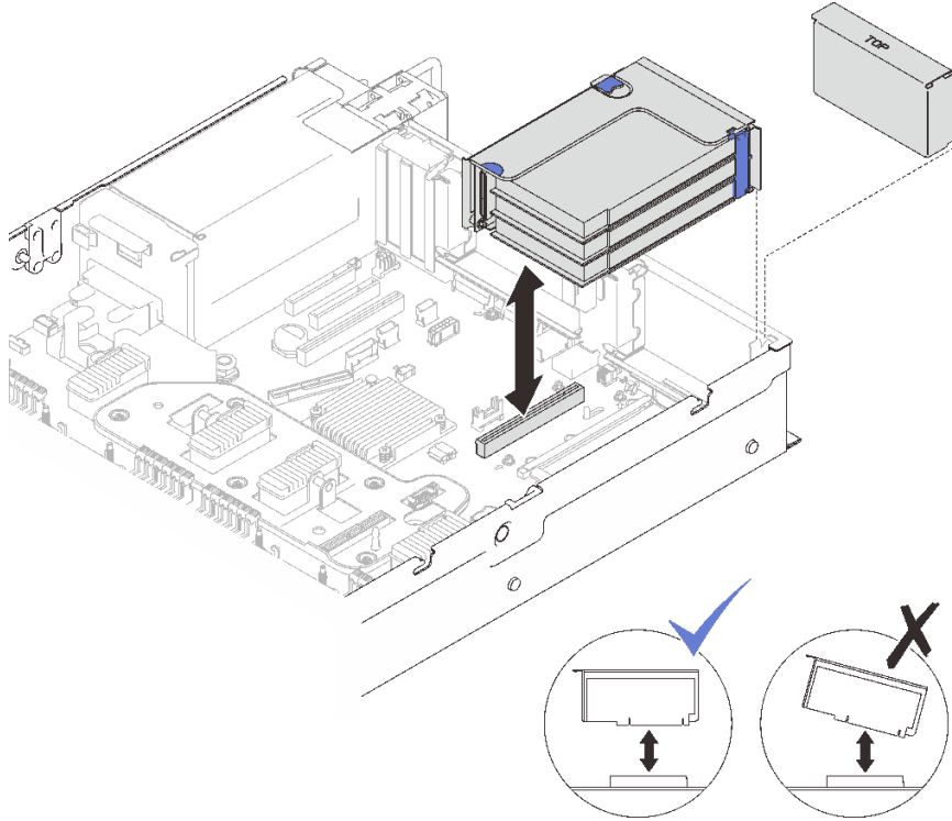
그림 68. 영역 1에 PCIe 라이저 어셈블리 설치
