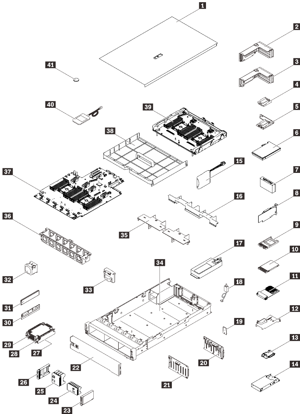
그림 17. 서버 구성 요소
