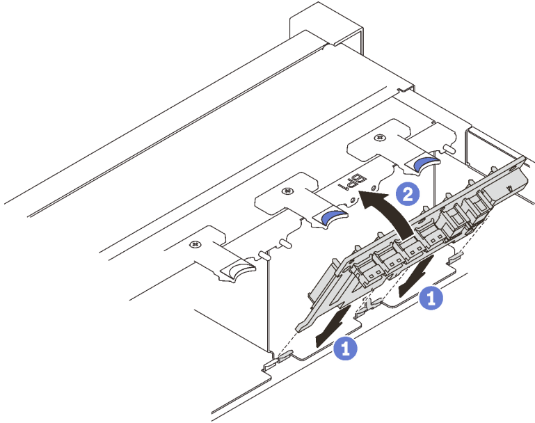
그림 55. 드라이브 백플레인 설치
