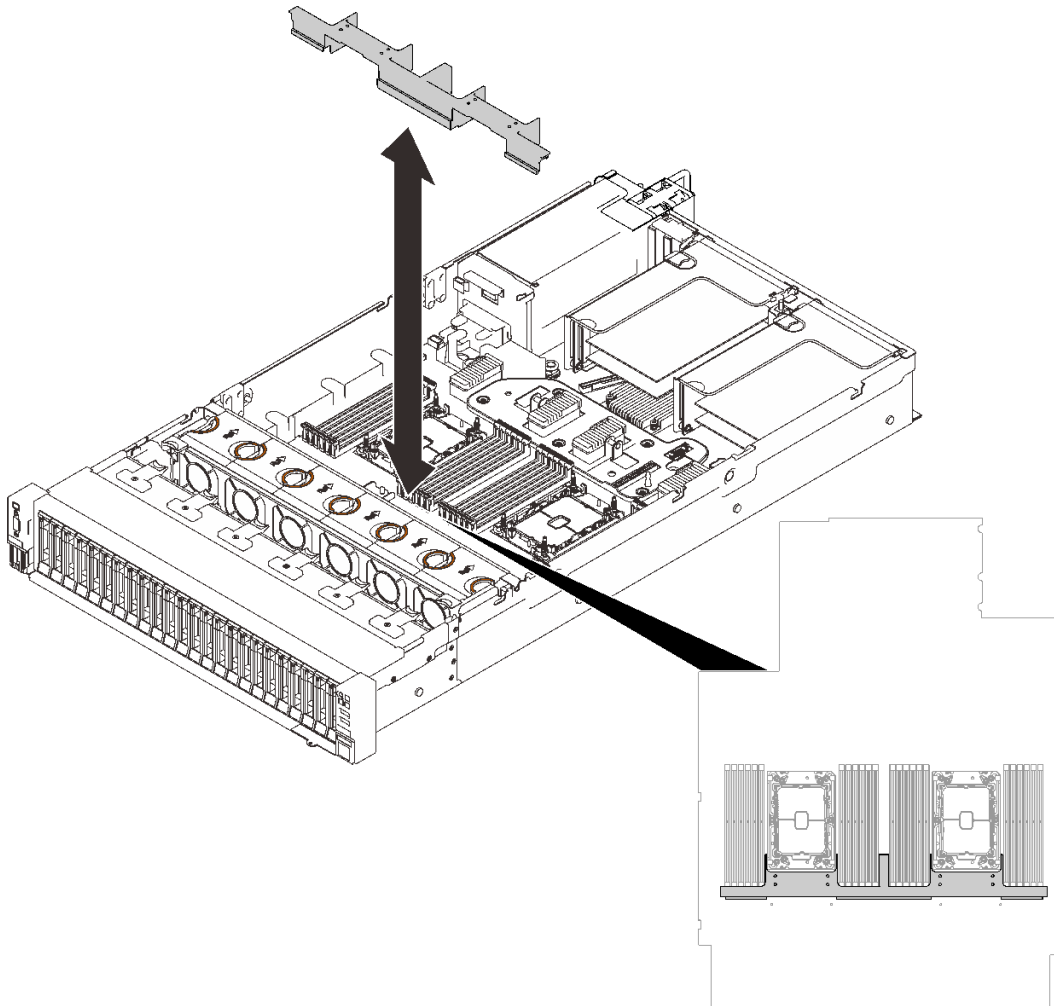
그림 21. 확장 트레이 공기 조절 장치 설치
