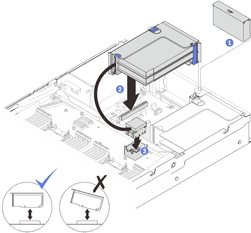
그림 70. 영역 2에 PCIe 라이저 어셈블리 설치
