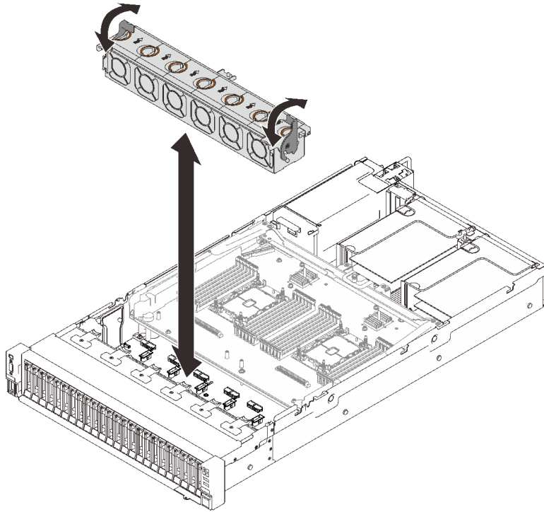
그림 54. 팬 케이스 어셈블리 제거
