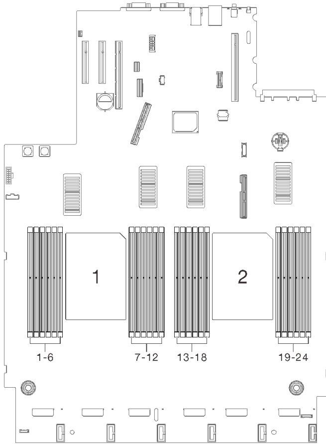
그림 76. 시스템 보드의 프로세서 1 및 2 위치
