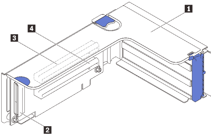
그림 38. x16/x16 PCIe 라이저 카드 커넥터
