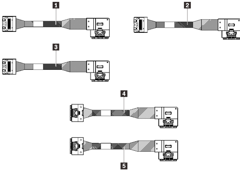
그림 31. SAS/SATA 케이블 키트
