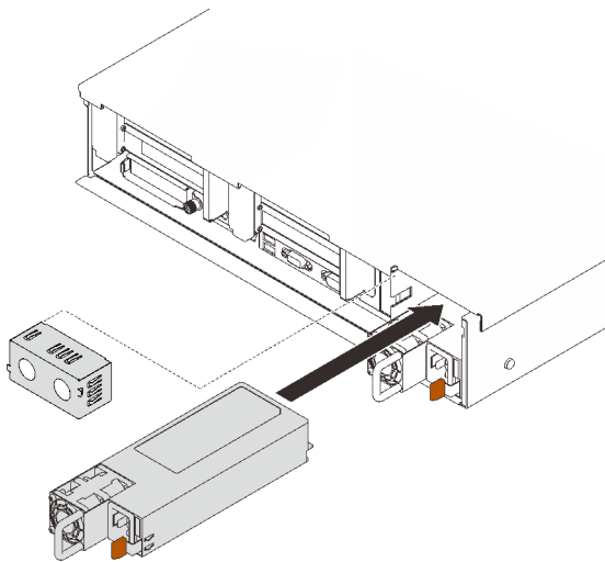
그림 50. 전원 공급 장치 설치
