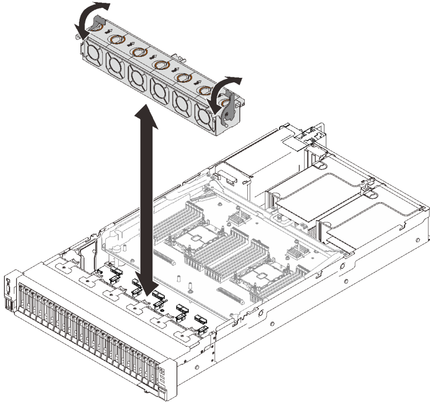
그림 87. 팬 케이스 어셈블리 장착
