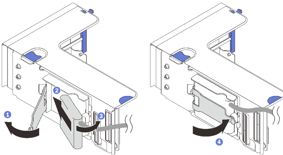
그림 63. 플래시 전원 모듈 설치
