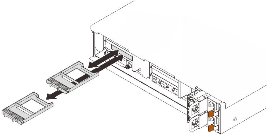
그림 45. 7mm 드라이버 필러 제거
