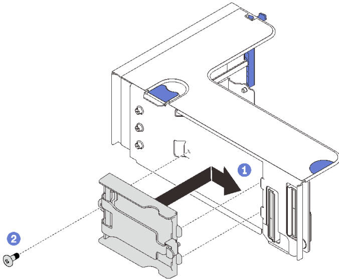
그림 62. 수직 홀더 설치 중
