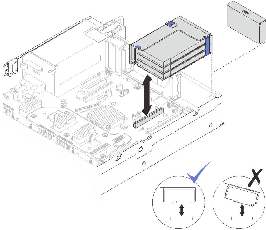
그림 57. 영역 1에서 PCIe 라이저 어셈블리 제거
