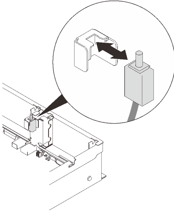
그림 56. 침입 스위치 설치
