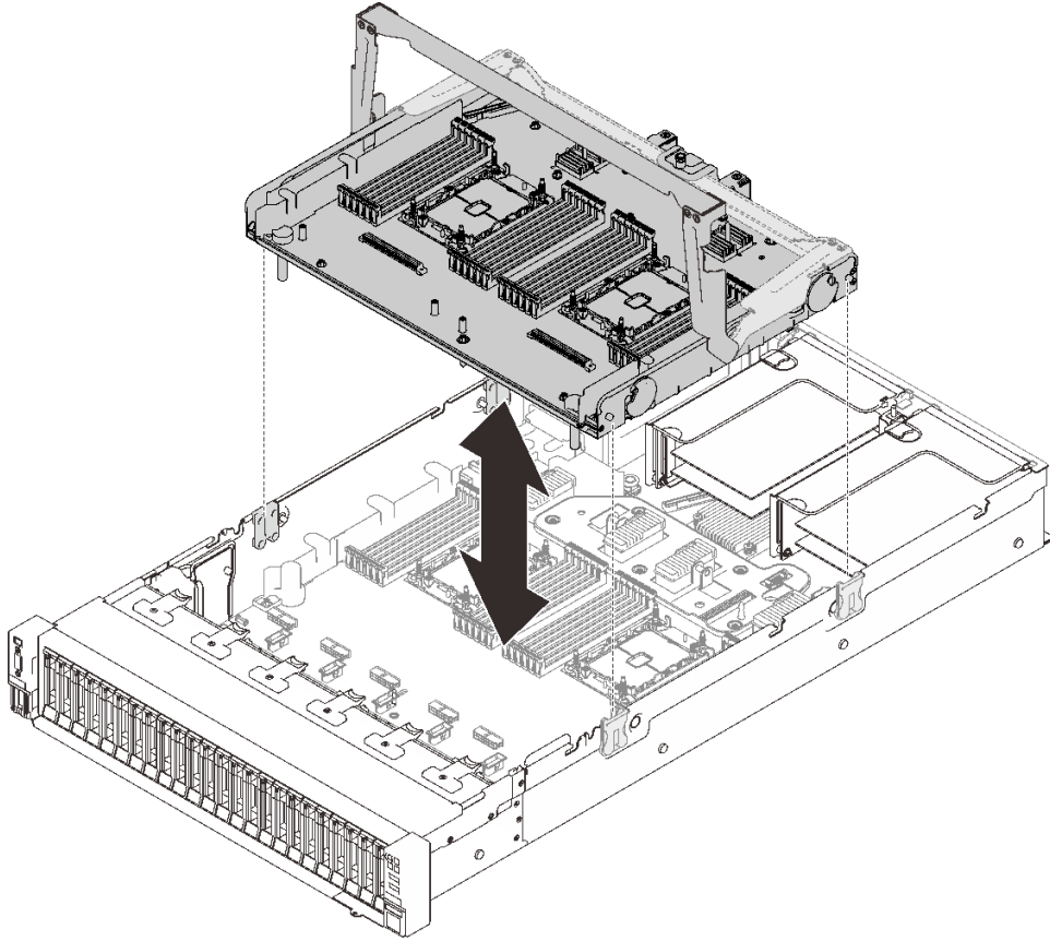
그림 84. 프로세서 및 메모리 확장 트레이 설치
