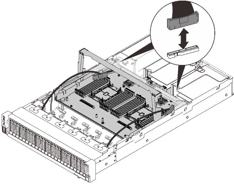
그림 23. 확장 트레이에 케이블 연결
