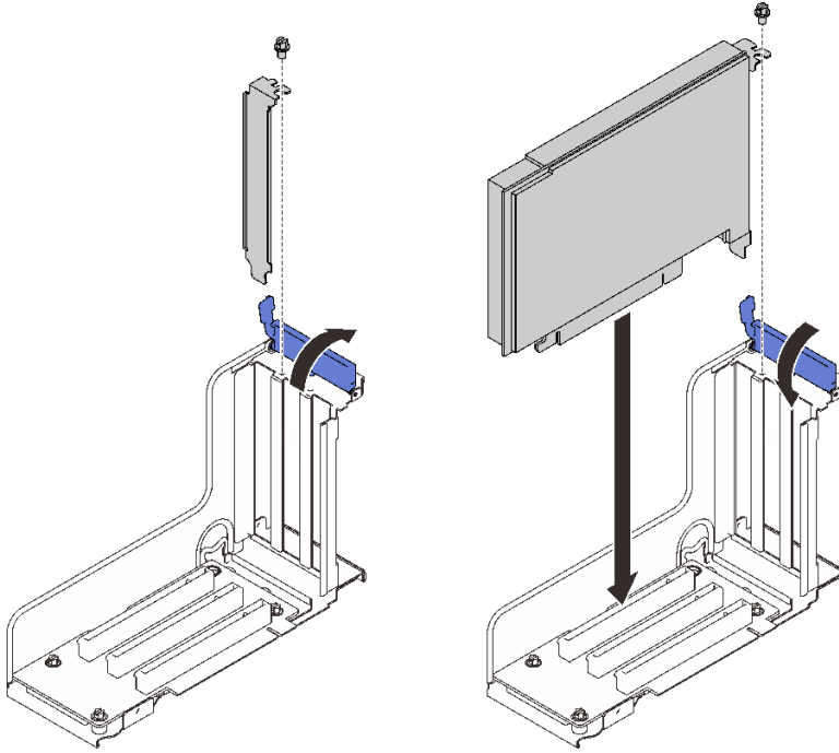
그림 60. PCIe 라이저 어셈블리에 어댑터 설치
