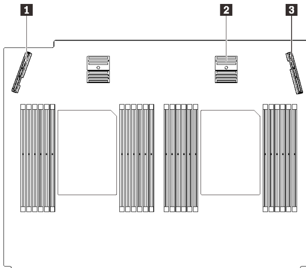
그림 44. 프로세서 및 메모리 확장 트레이 커넥터
