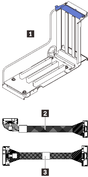
그림 39. x16/x16/x16 PCIe 라이저 카드
