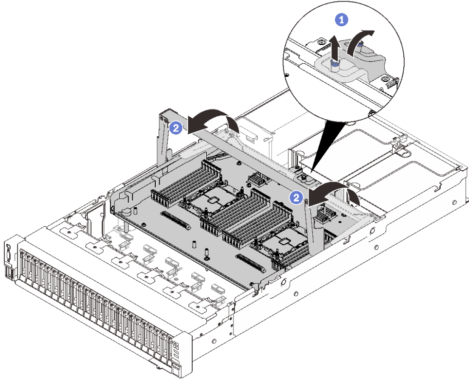
그림 72. 프로세서 및 메모리 확장 트레이 분리
