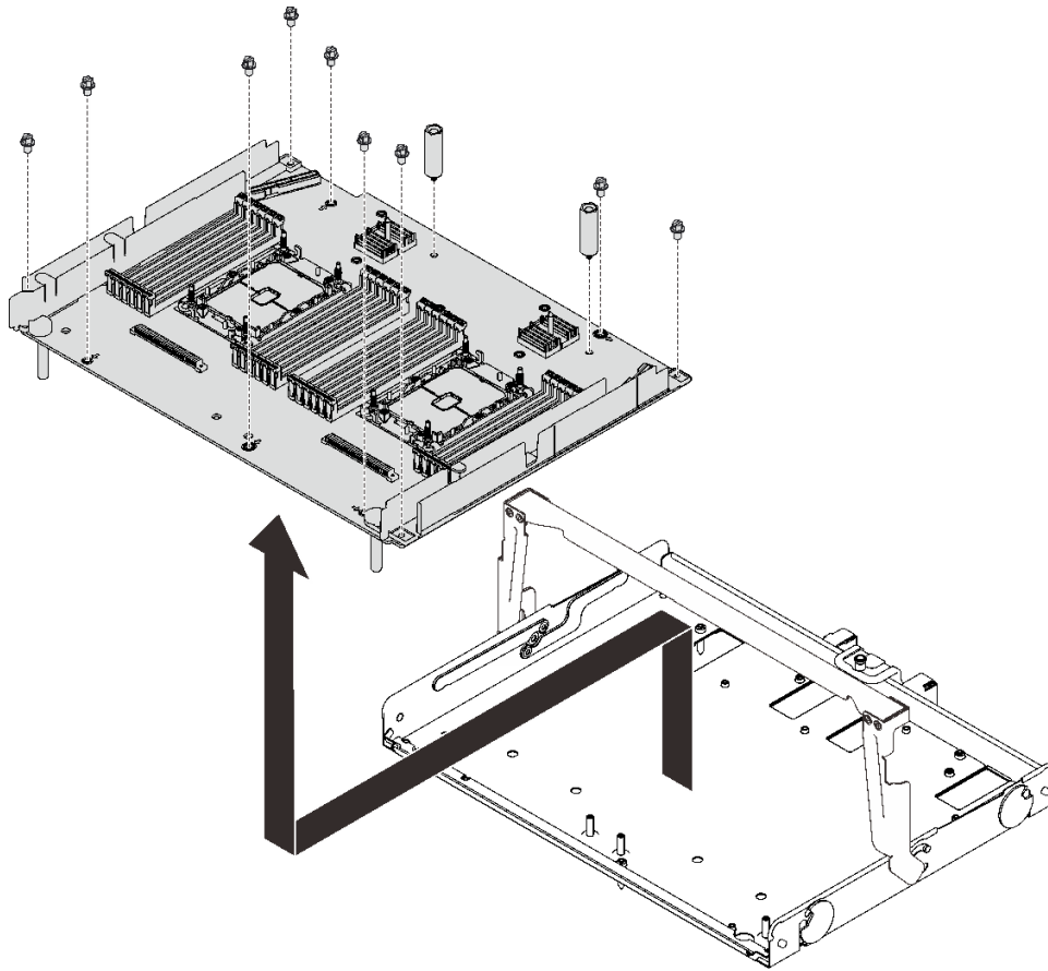
그림 75. 확장 트레이 분해
