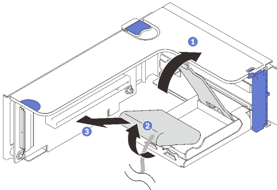
图 53. 从垂直夹持器上卸下快速充电模块
