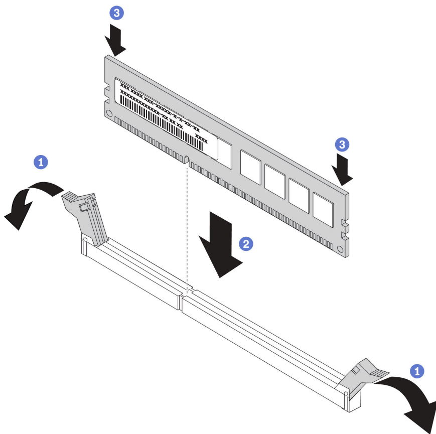
图 71. 安装内存条
