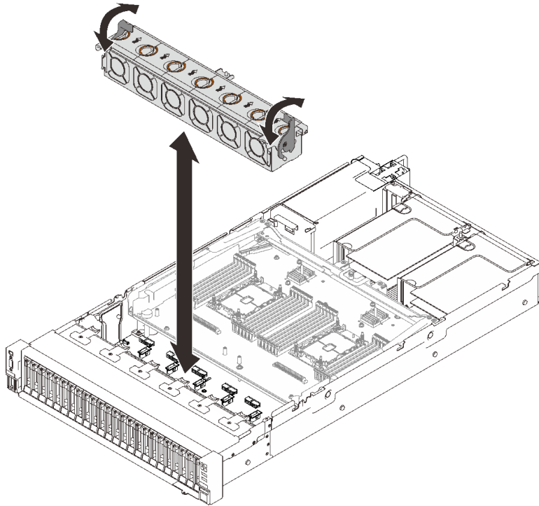
图 49. 卸下风扇架组合件
