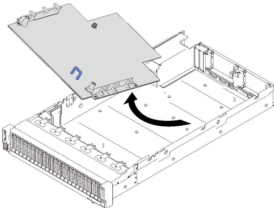
图 125. 卸下主板
