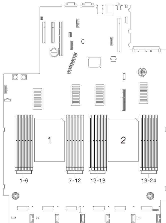
图 102. 主板上的处理器 1 和 2 位置
