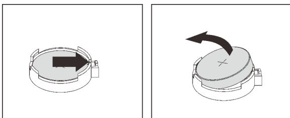
图 44. 卸下 CMOS 电池
