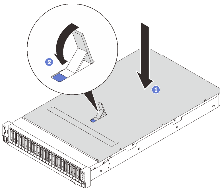
图 131. 安装顶盖
