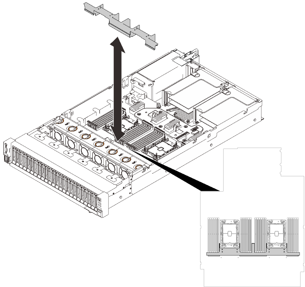
图 61. 卸下扩展托盘导风罩
