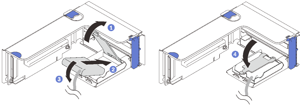
图 58. 将快速充电模块安装到水平夹持器中
