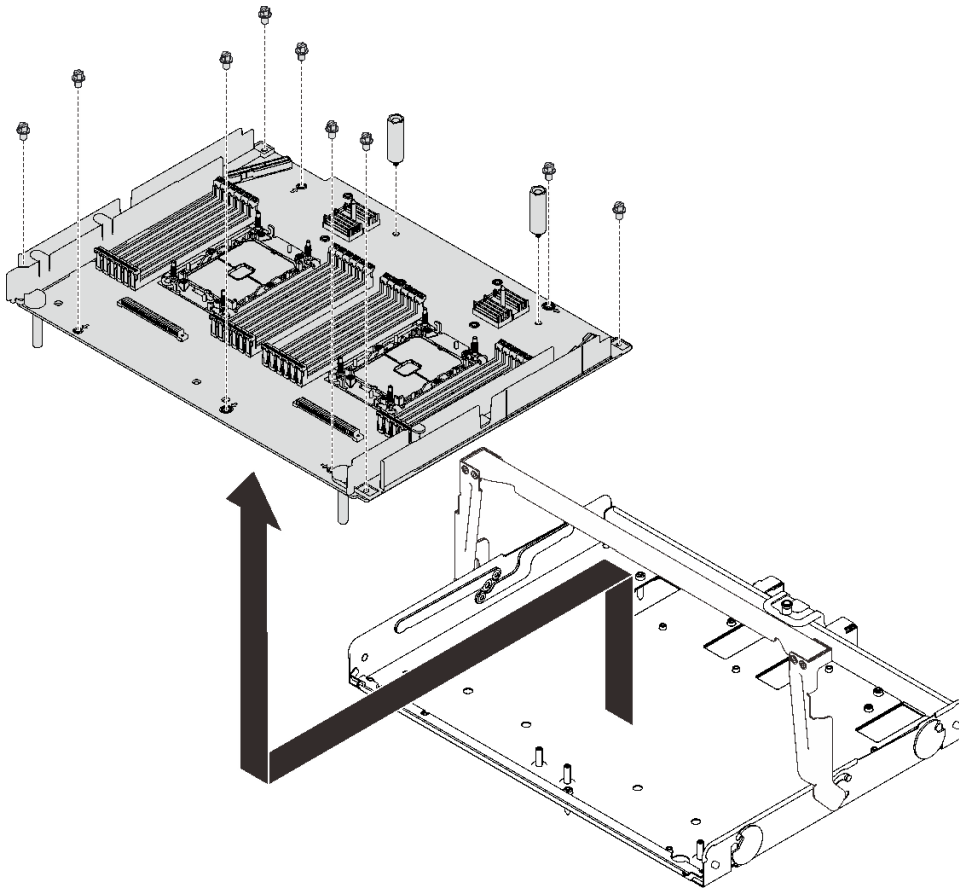
图 113. 拆卸扩展托盘
