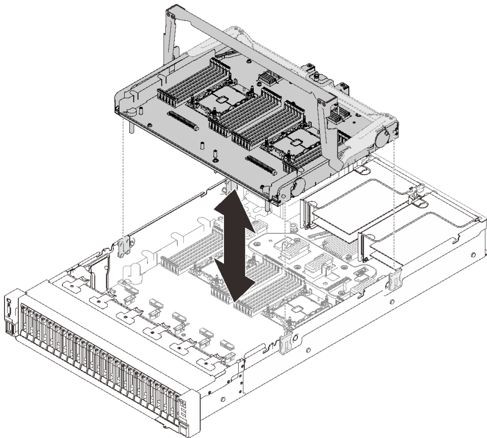
图 112. 卸下处理器和内存扩展托盘
