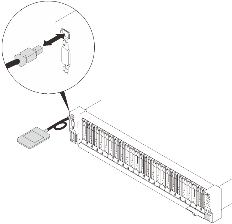
图 47. 连接外部 LCD 诊断手持设备线缆
