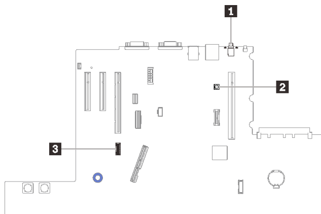
图 17. 开关、跳线和按钮
