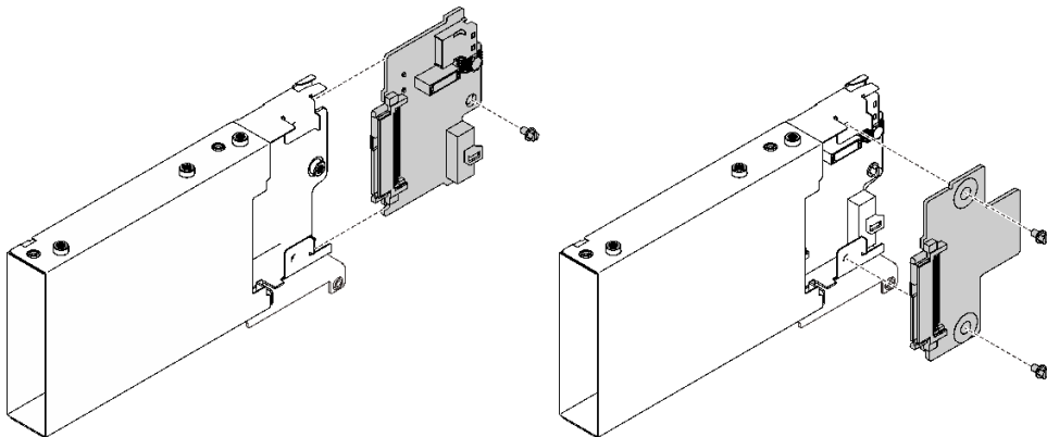
图 37. 拆卸 7 毫米硬盘仓
