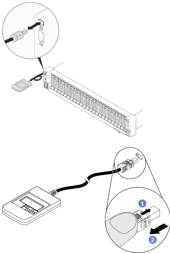
图 46. 拔下外部 LCD 诊断手持设备线缆
