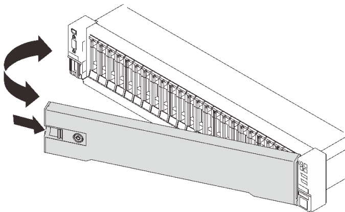
图 120. 安装安全挡板
