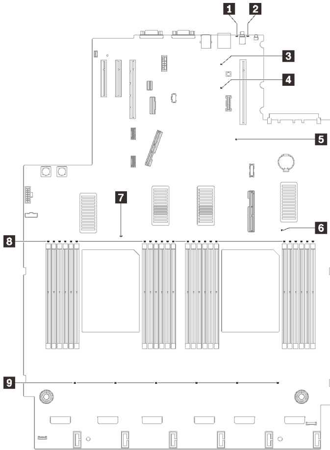
图 18. 主板 LED
