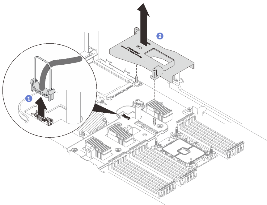
图 42. 卸下 OCP 适配器导风罩
