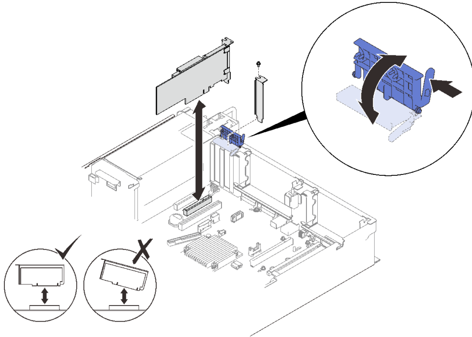
图 77. 从主板上卸下适配器
