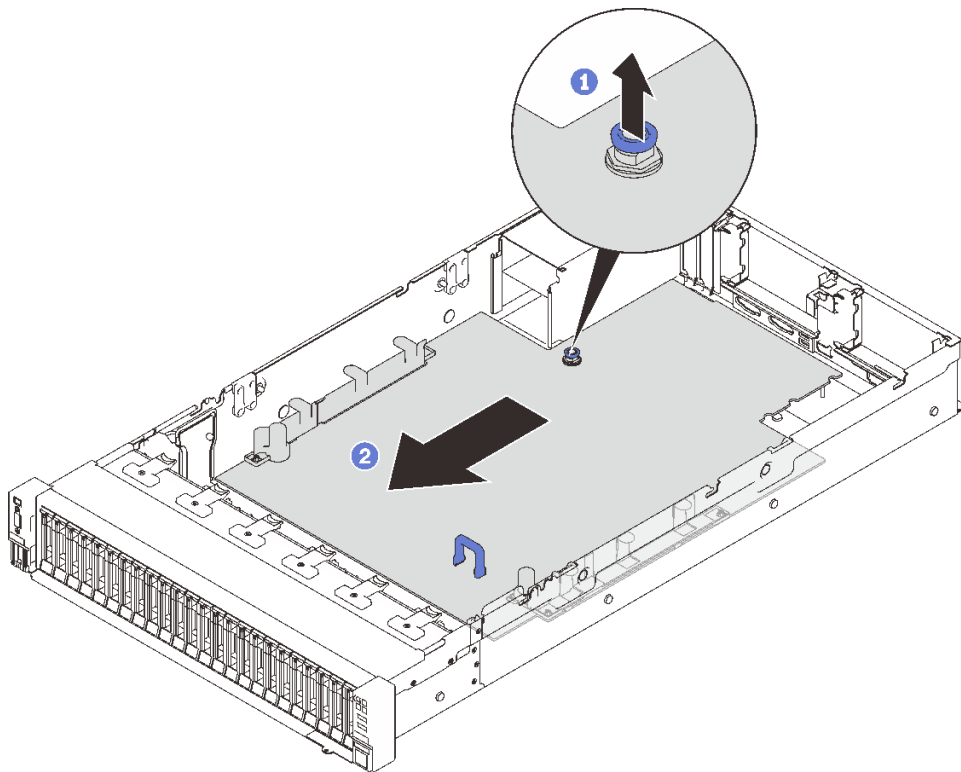
图 124. 拆卸主板
