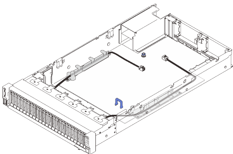
图 22. 主板上的线缆导轨
