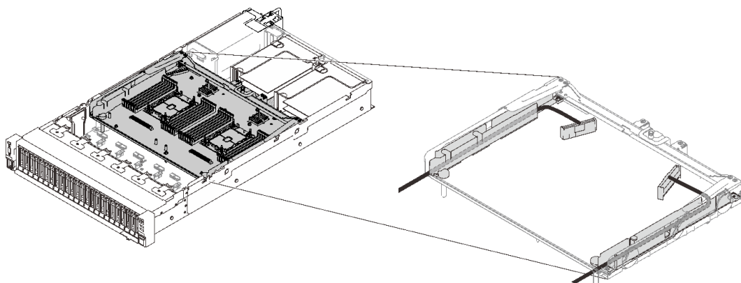
图 23. 处理器和内存扩展托盘上的线缆导轨
