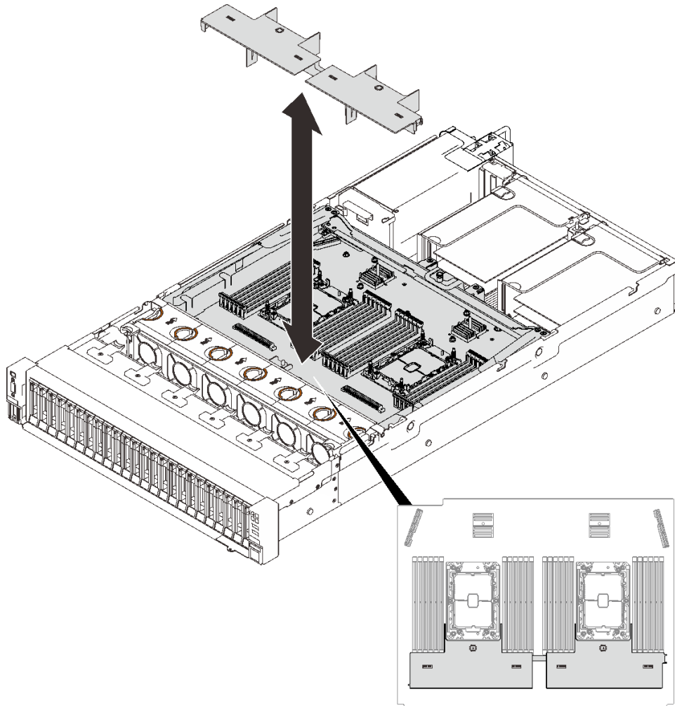
图 134. 将导风罩安装到扩展托盘
