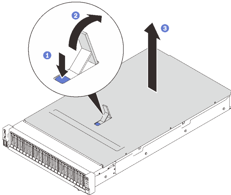
图 130. 卸下顶盖
