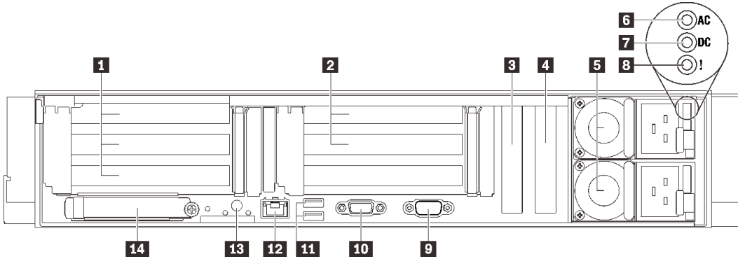
图 6. 后视图
