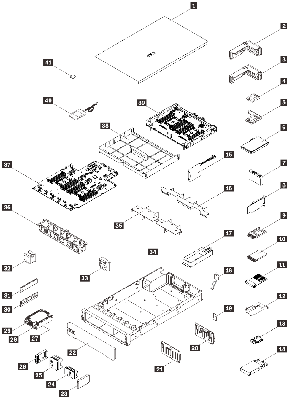
图 20. 服务器组件
