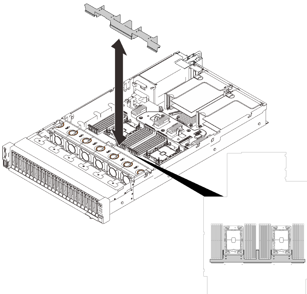
图 114. 安装扩展托盘导风罩
