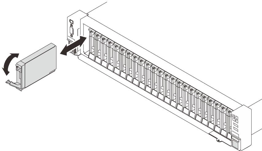
图 33. 安装 2.5 英寸硬盘
