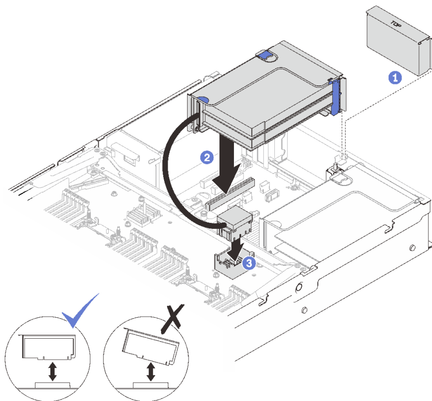
图 83. 将 PCIe 转接卡组合件安装到区域 2
