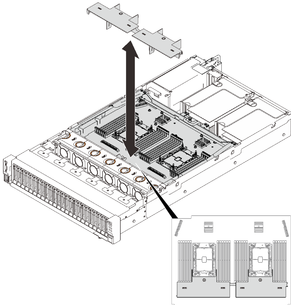
图 60. 从扩展托盘上卸下导风罩
