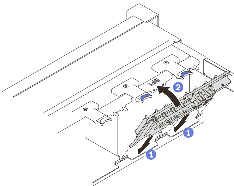
图 31. 安装硬盘背板
