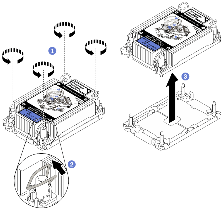
图 99. 卸下 PHM
