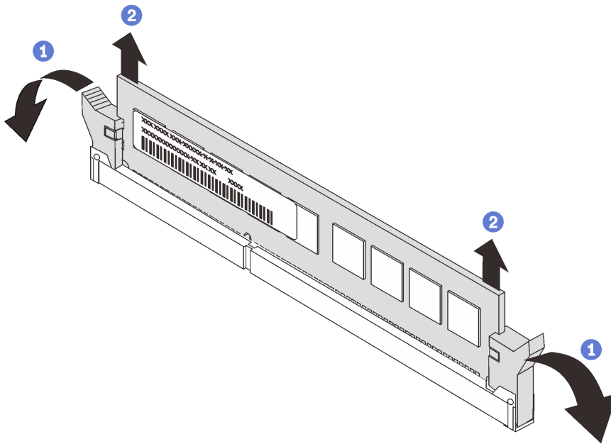
图 70. 卸下内存条
