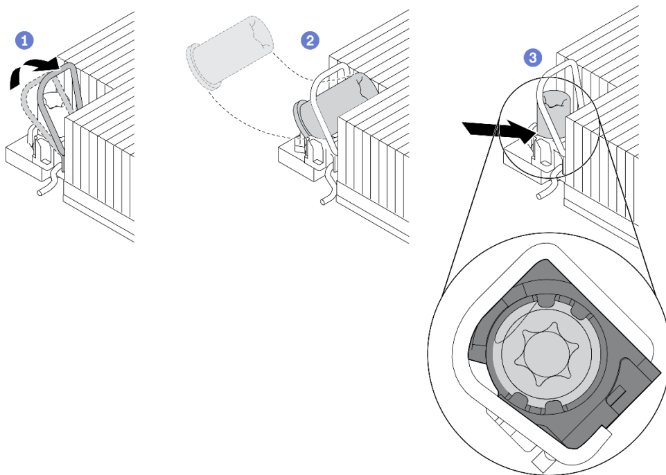
图 63. 将内六角 T30 螺母安装到散热器中
