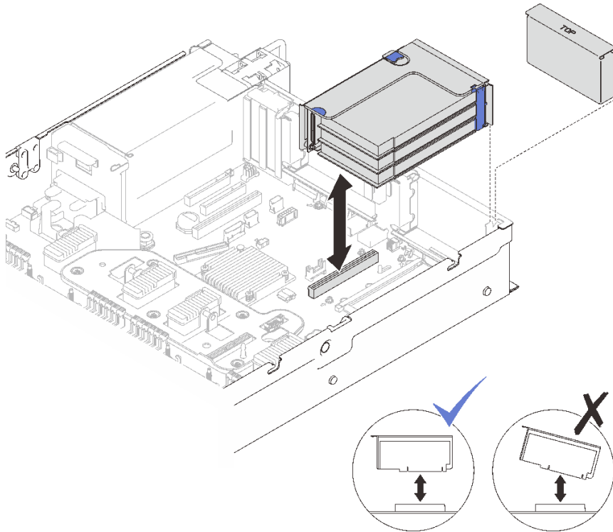
图 74. 从区域 1 中卸下 PCIe 转接卡组合件
