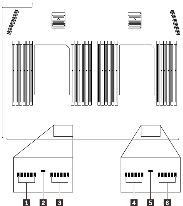
图 19. 处理器和内存扩展托盘 LED
