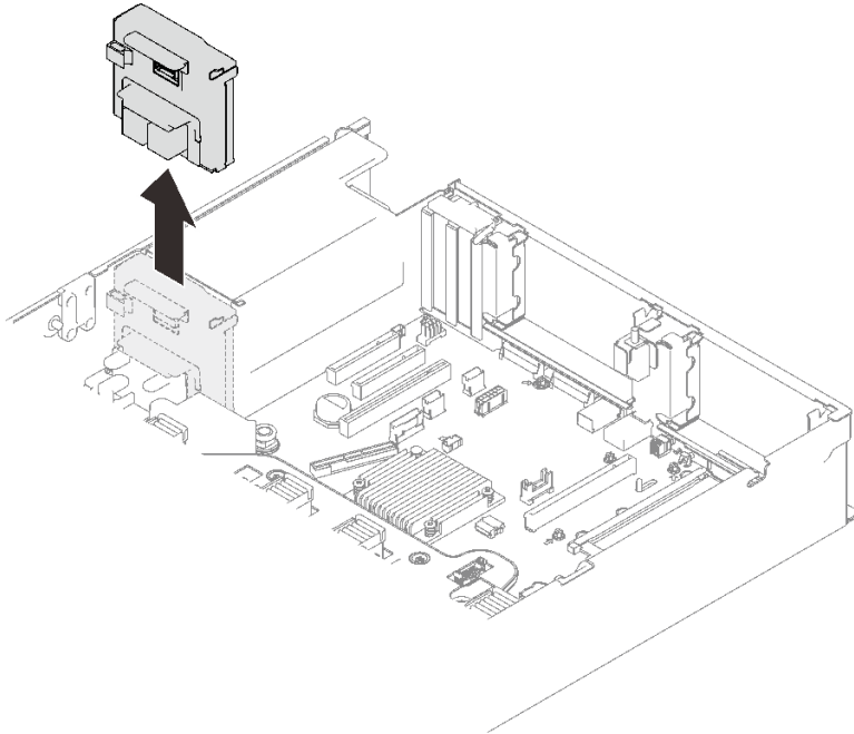
图 85. 卸下电源背板
