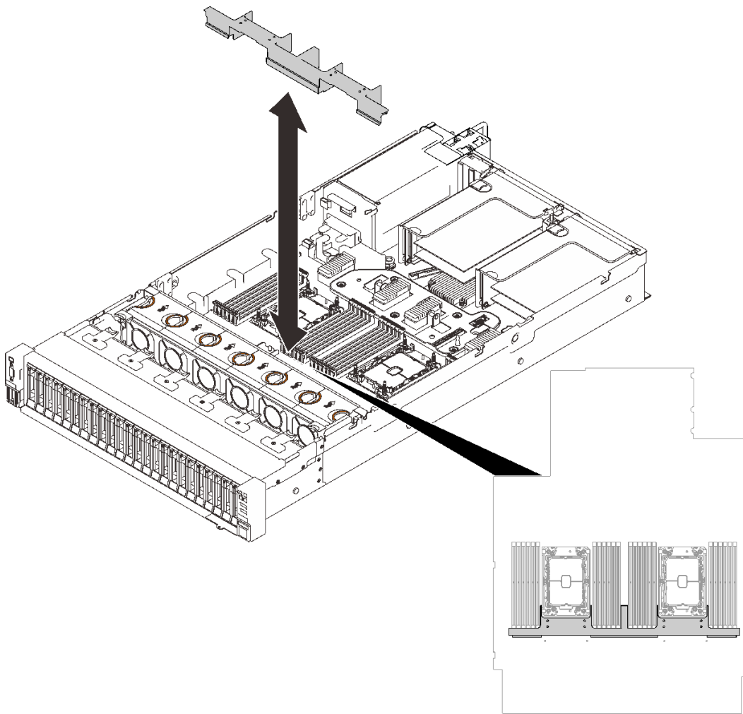
图 24. 安装扩展托盘导风罩
