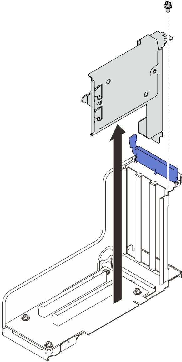
图 56. 从 PCIe 转接卡上卸下来夹持器支架
