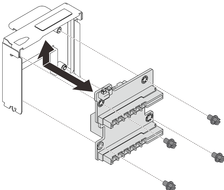
图 86. 拆卸电源背板
