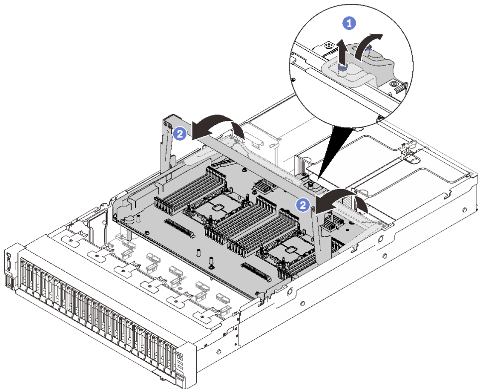
图 110. 拆卸处理器和内存扩展托盘
