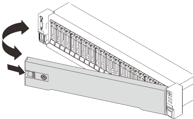
图 119. 卸下安全挡板
