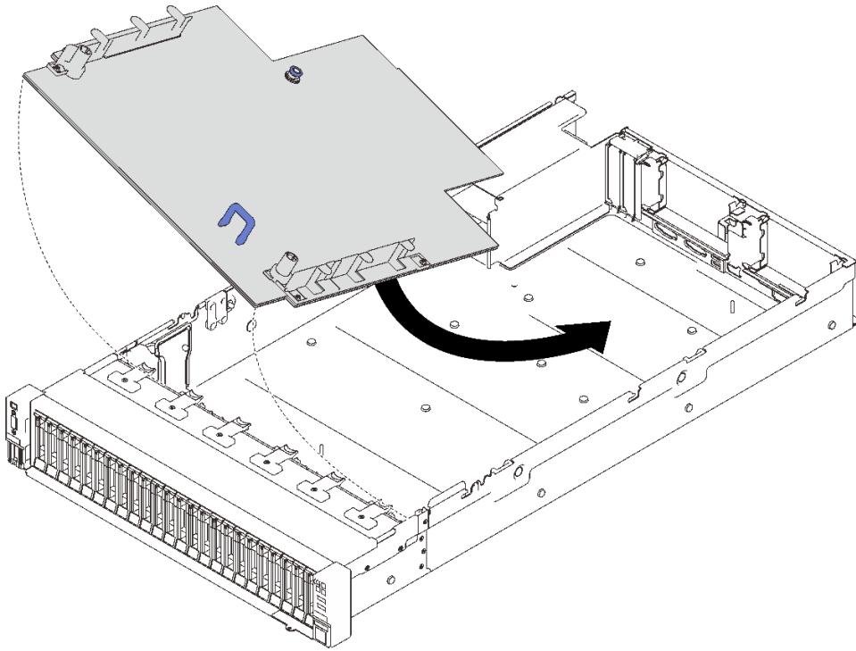
图 127. 安装主板
