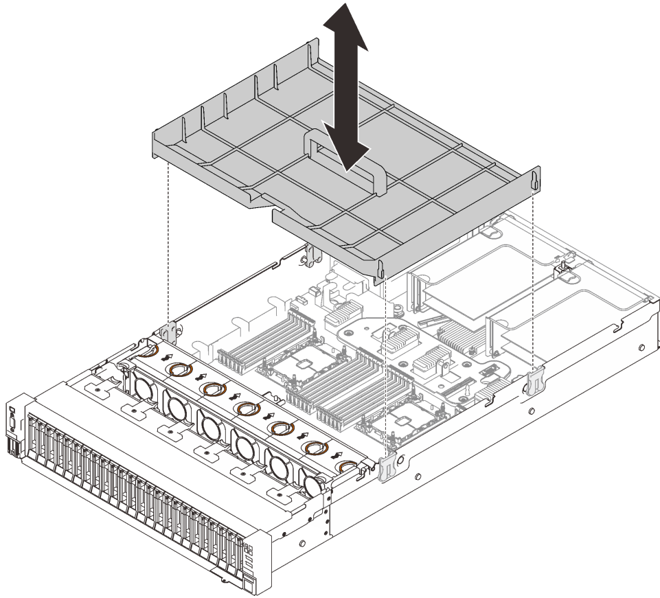
图 122. 卸下主板导风罩
