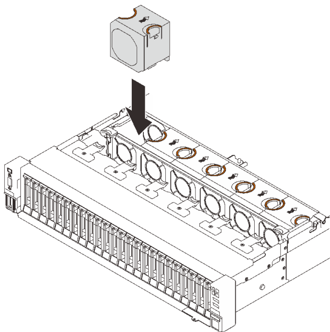
图 52. 安装风扇
