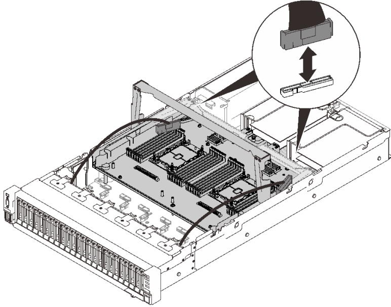
图 116. 将线缆连接到扩展托盘
