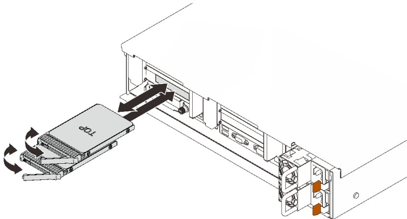
图 41. 安装 7 毫米硬盘
