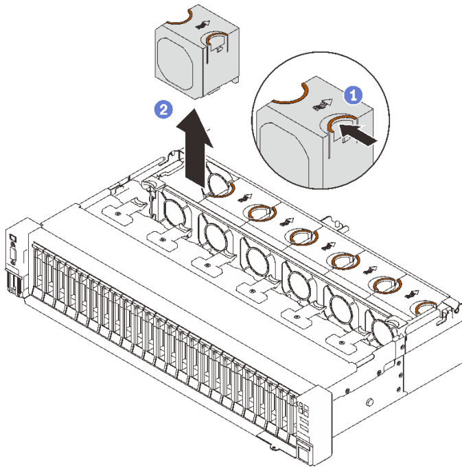
图 51. 卸下风扇
