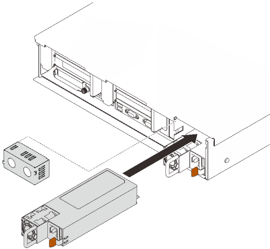
图 92. 安装电源模块单元
