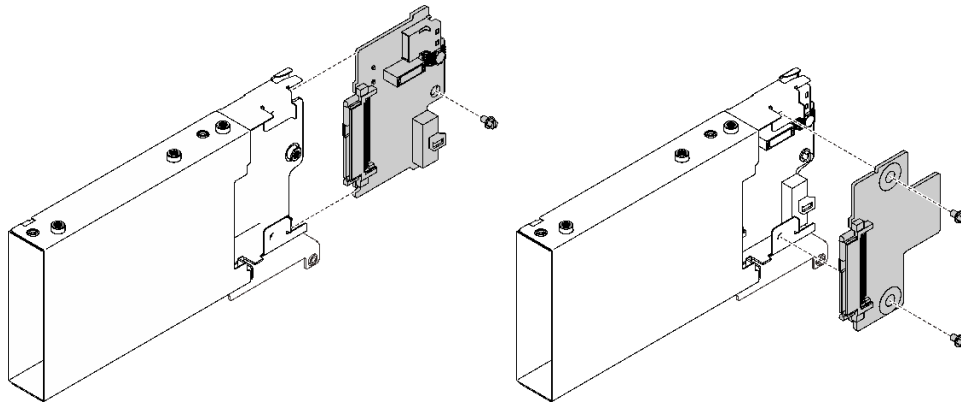
图 38. 安装 7 毫米硬盘背板
