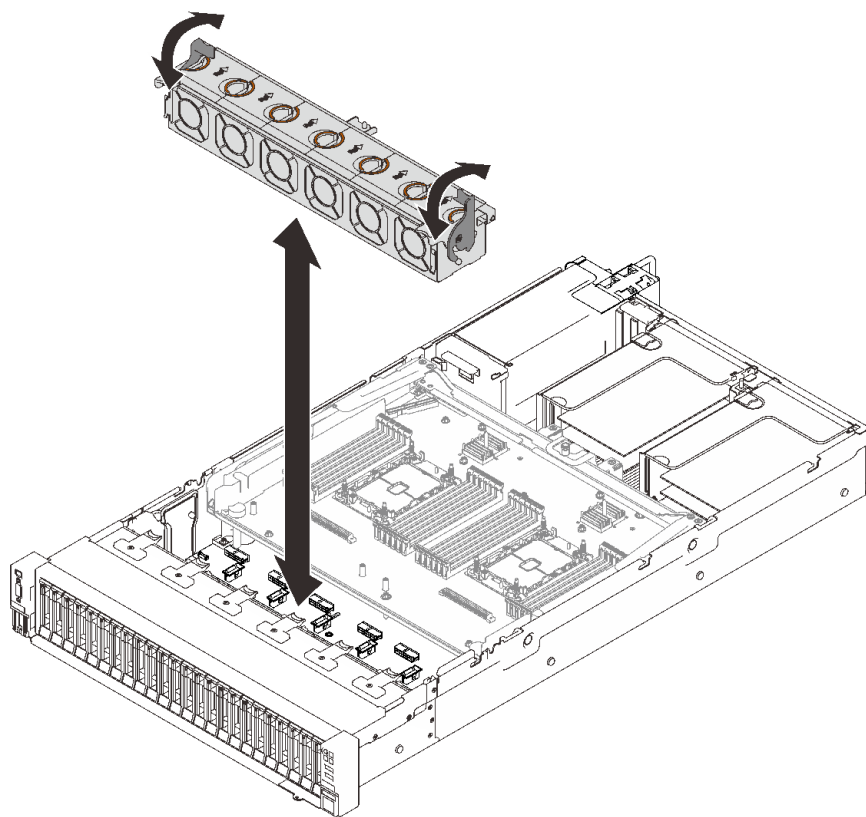
图 50. 安装风扇架组合件
