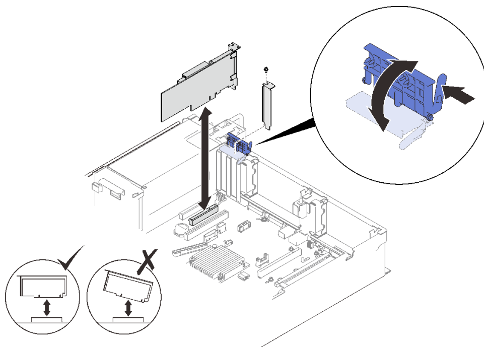
图 79. 将适配器安装到主板
