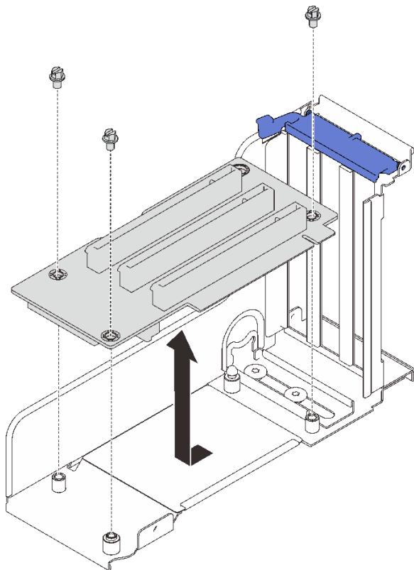
图 76. 拆卸 PCIe 转接卡
