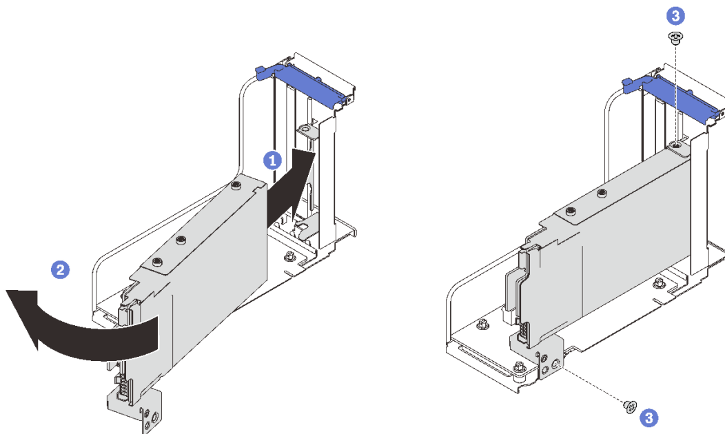
图 39. 将 7 毫米硬盘仓安装到转接卡
