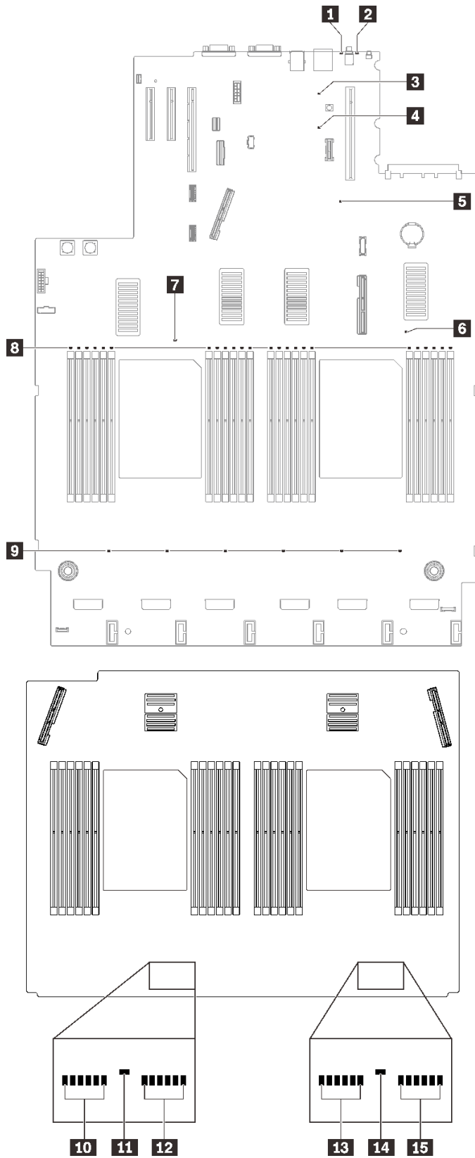
图 137. 主板和扩展板 LED
