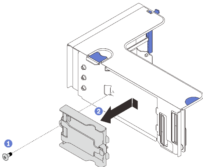
图 55. 卸下垂直夹持器
