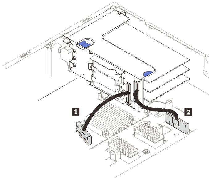
图 82. 将 PCIe 线缆从 x16/x16/x16 转接卡连接到主板
