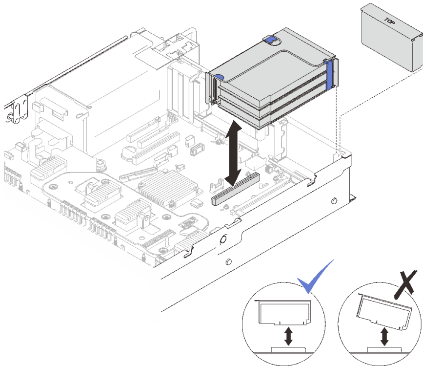
图 81. 将 PCIe 转接卡组合件安装到区域 1
