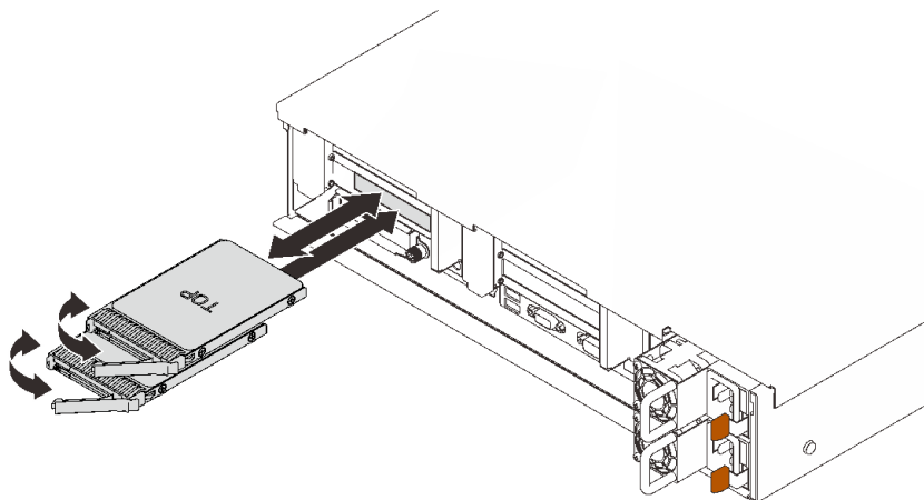
图 34. 卸下 7 毫米硬盘
