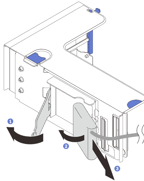
图 54. 从水平夹持器上卸下快速充电模块
