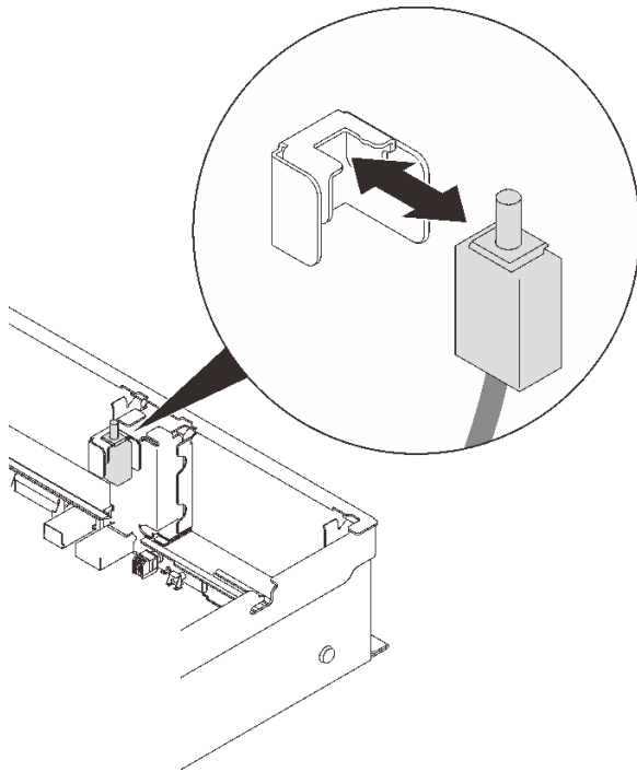
图 65. 安装入侵感应开关
