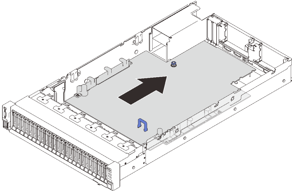
图 128. 安装主板
