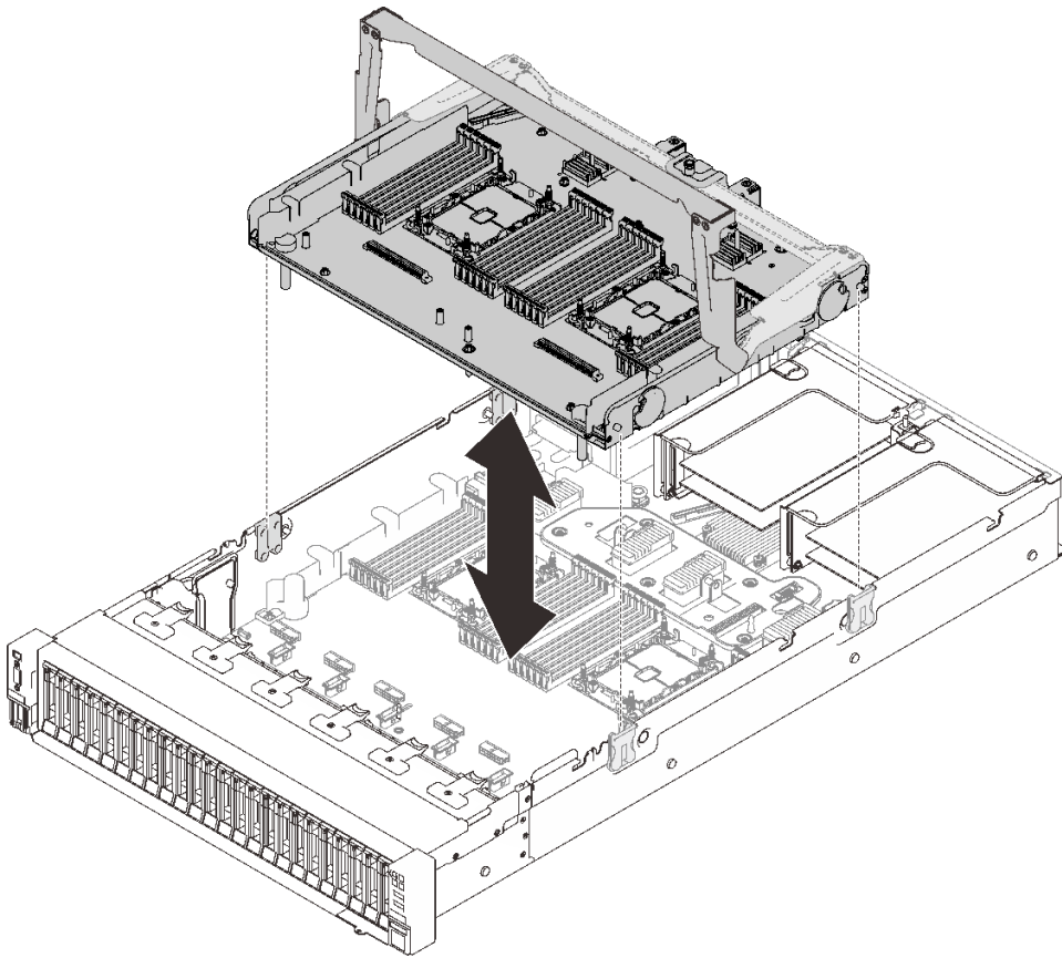
图 115. 安装处理器和内存扩展托盘
