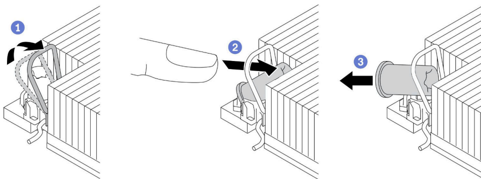
图 62. 从散热器上卸下内六角 T30 螺母
