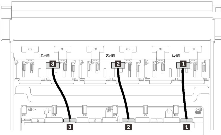
图 21. 硬盘背板电源线
