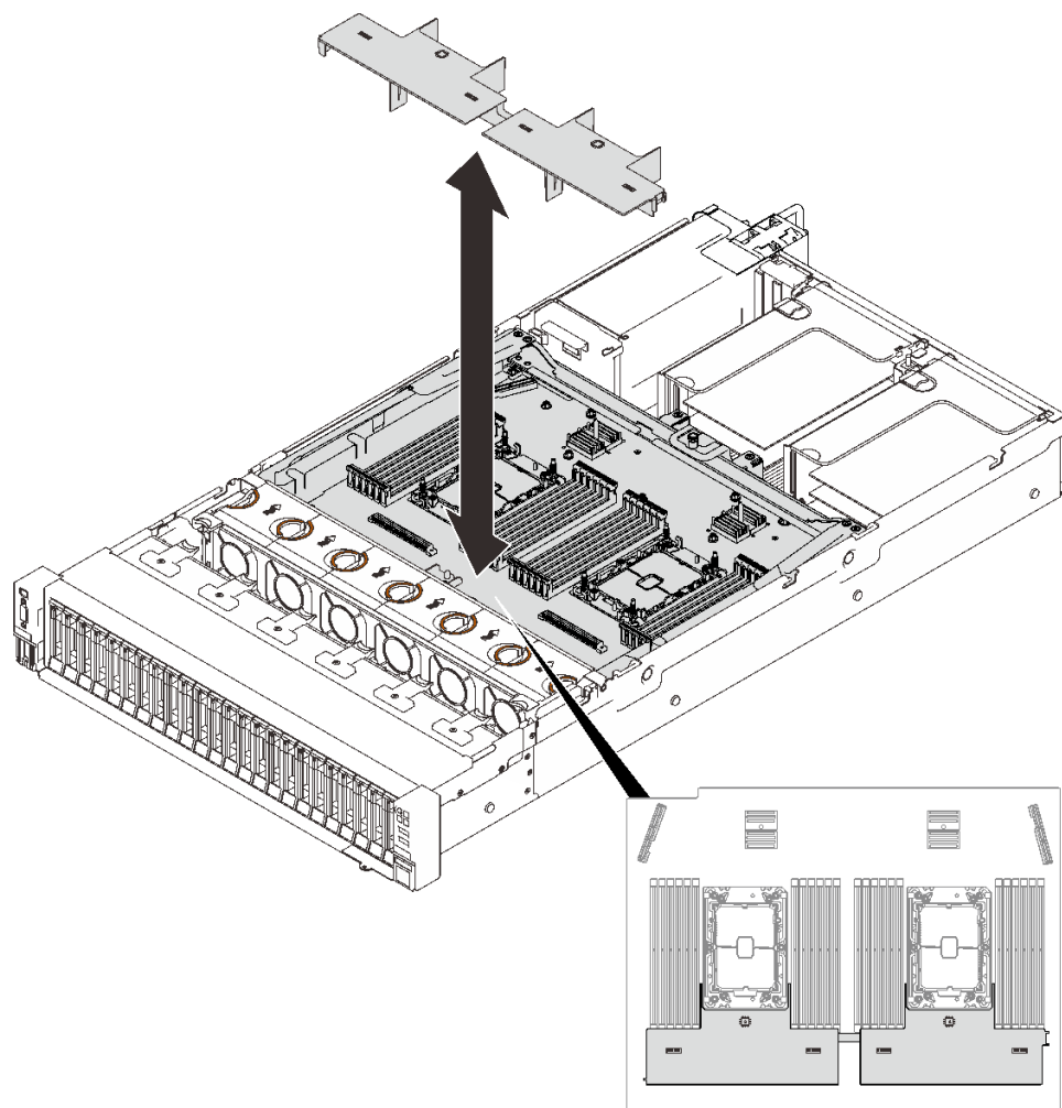
图 96. 从扩展托盘上卸下导风罩
