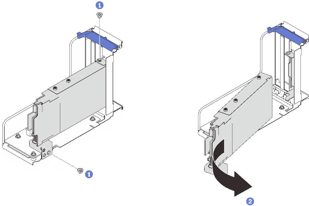
图 36. 从转接卡上卸下 7 毫米硬盘仓
