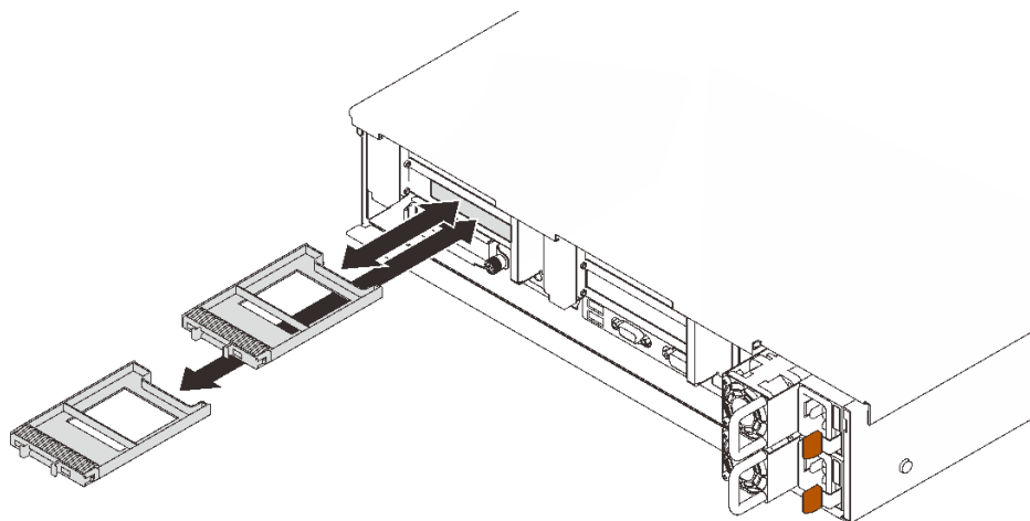
图 35. 安装 7 毫米硬盘填充件
