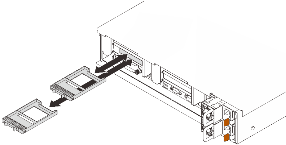
图 40. 卸下 7 毫米硬盘填充件
