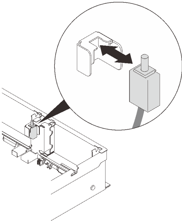
图 64. 卸下入侵感应开关
