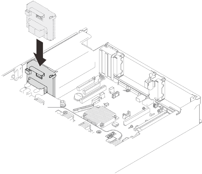
图 87. 安装电源背板
