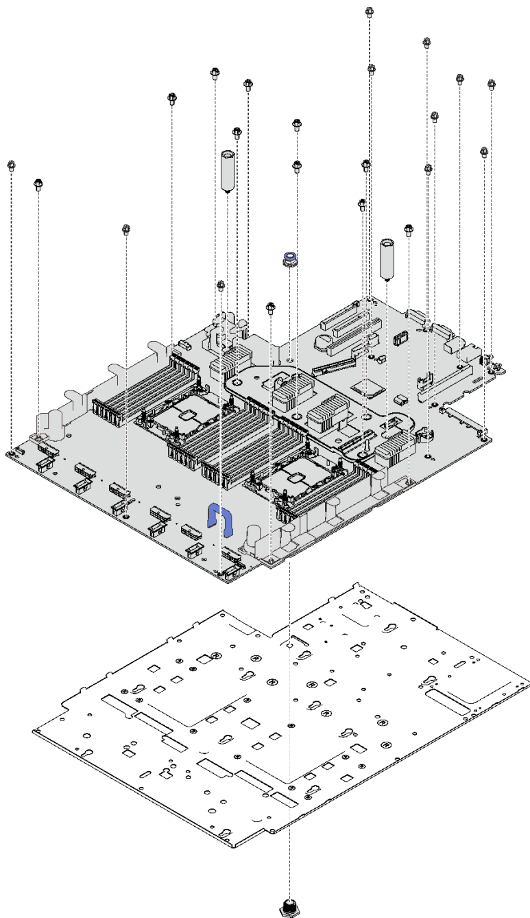
图 126. 拆卸主板
