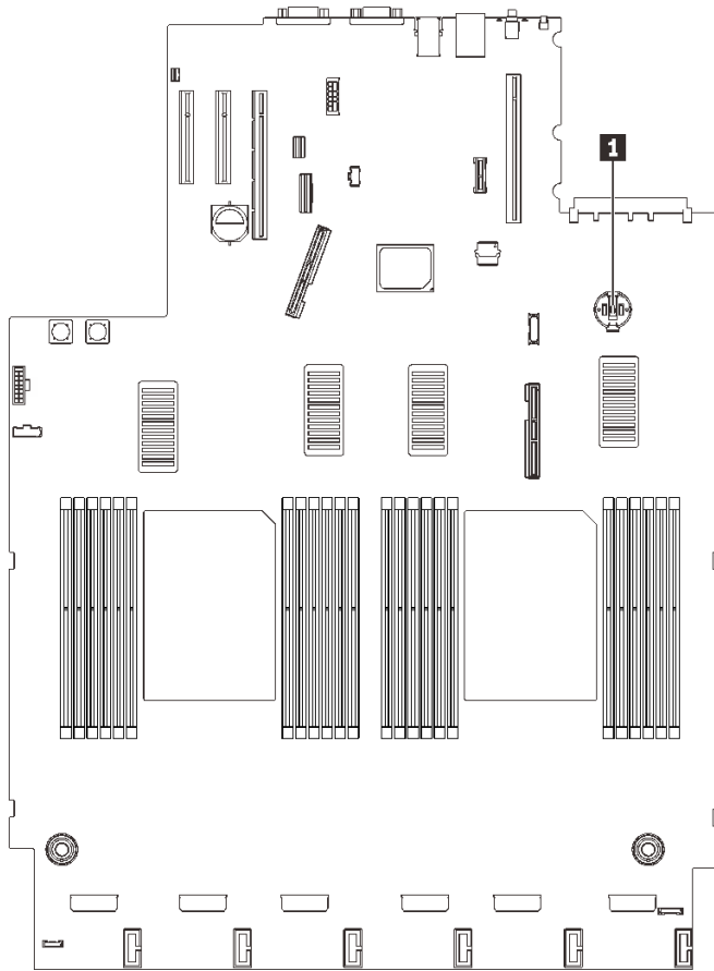
图 43. 主板上的 CMOS 电池位置
