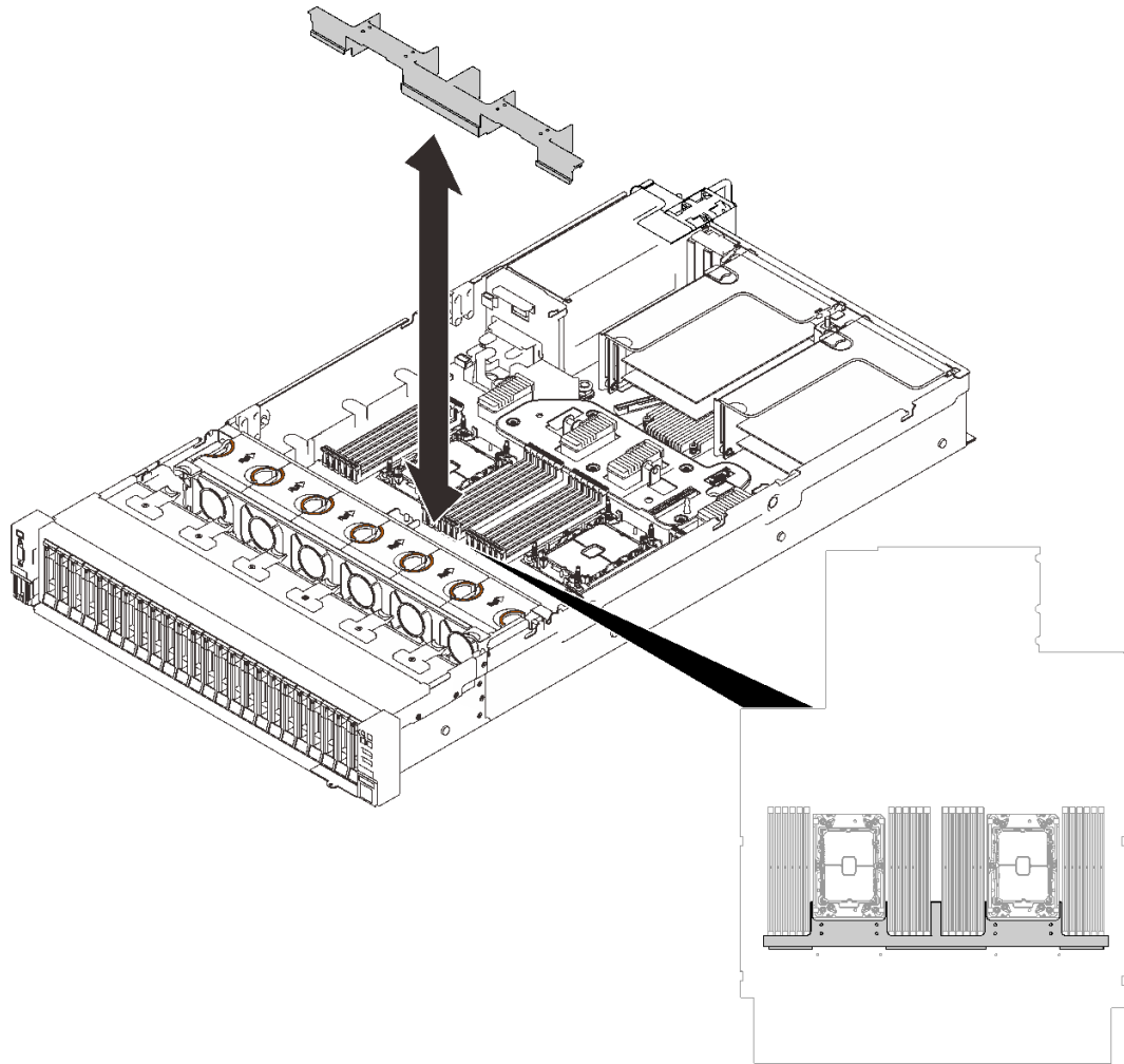
图 97. 卸下扩展托盘导风罩
