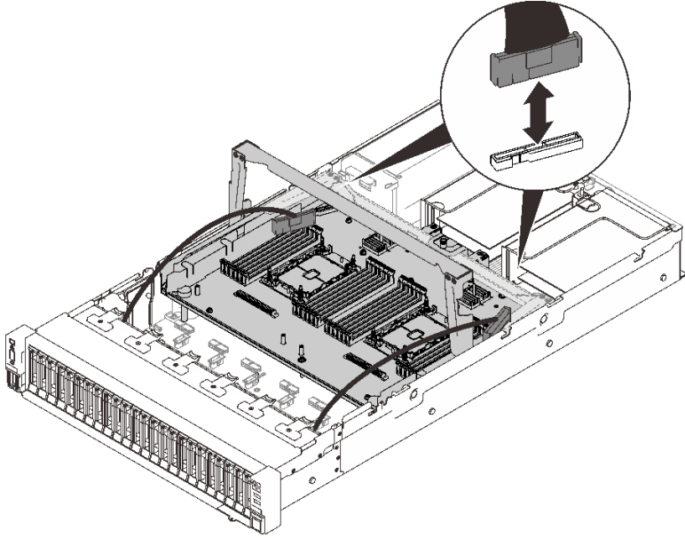
图 111. 拔下 PCIe 线缆
