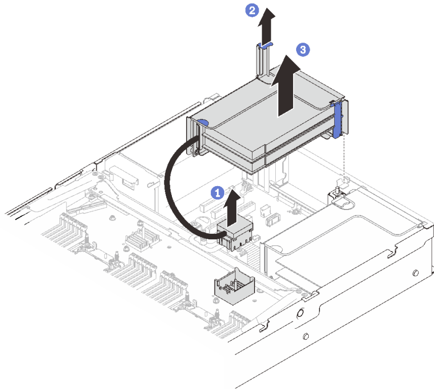
图 75. 从区域 2 中卸下 PCIe 转接卡组合件
