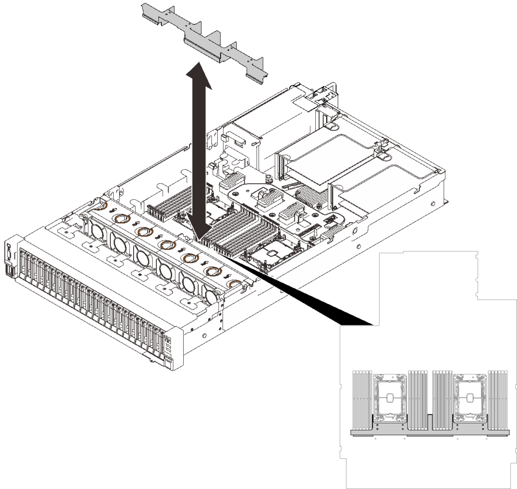
图 133. 将导风罩安装到主板
