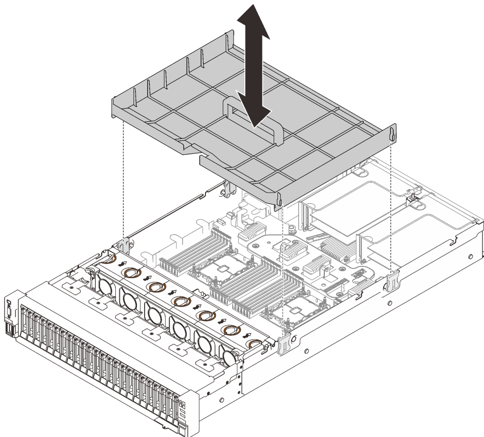
图 123. 安装主板导风罩
