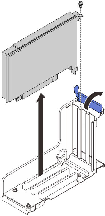
图 78. 从 PCIe 转接卡组合件中卸下适配器
