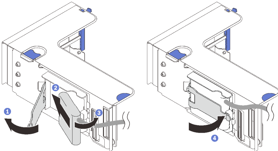
图 59. 将快速充电模块安装到垂直夹持器中
