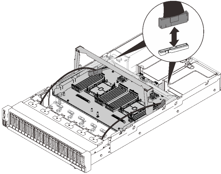
图 26. 将线缆连接到扩展托盘
