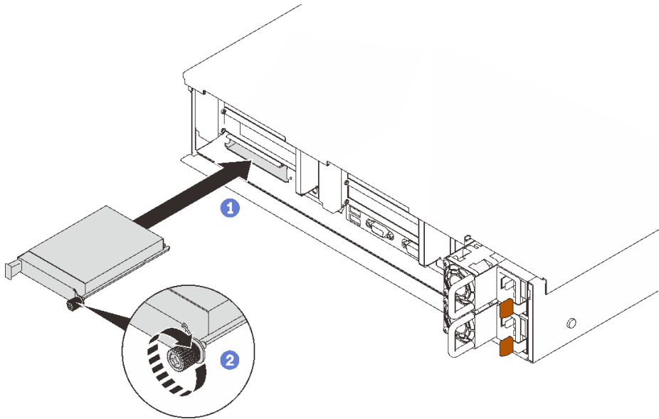
图 73. 安装 OCP 以太网适配器
