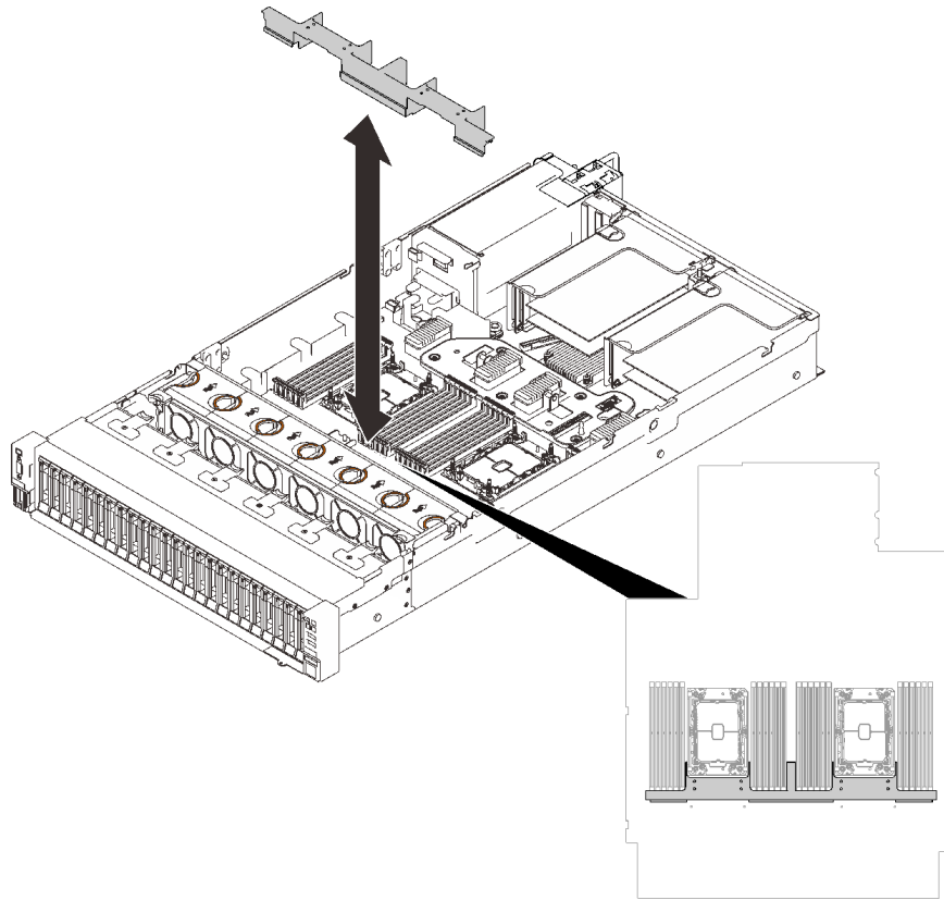
图 69. 卸下扩展托盘导风罩
