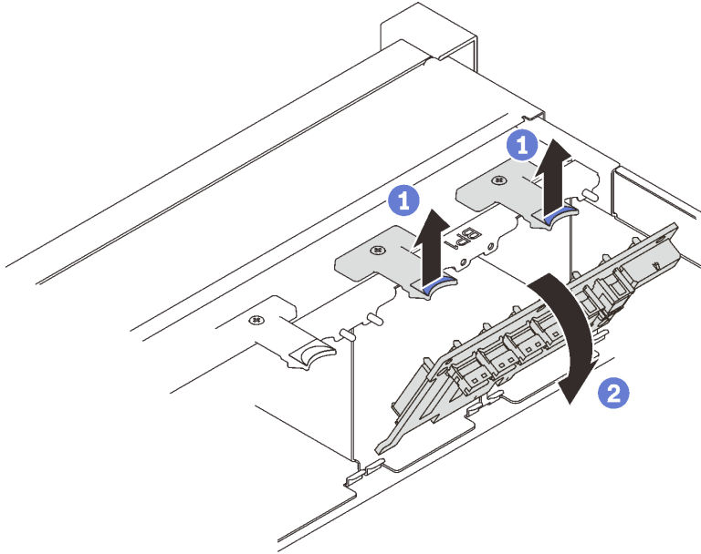
图 30. 卸下硬盘背板
