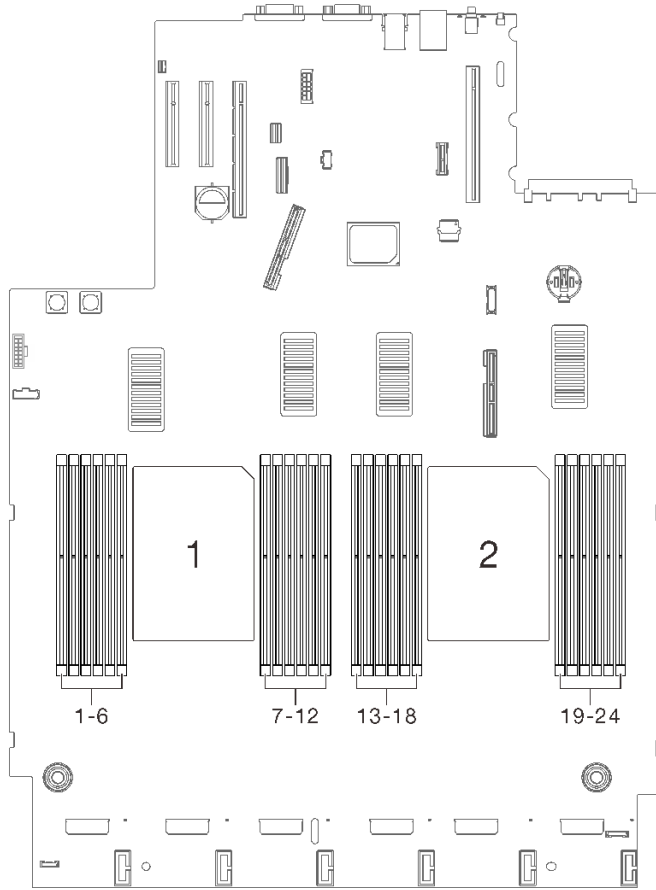
图 76. 主板上的处理器 1 和 2 位置
