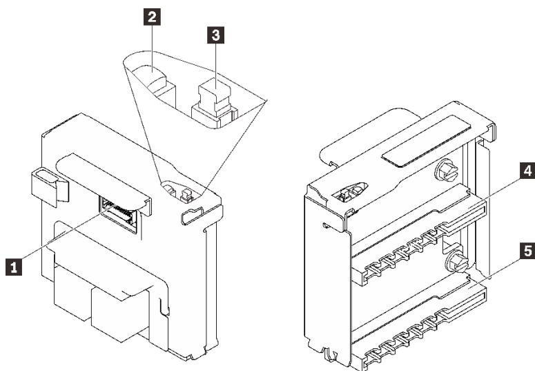
图 11. 电源背板组件
