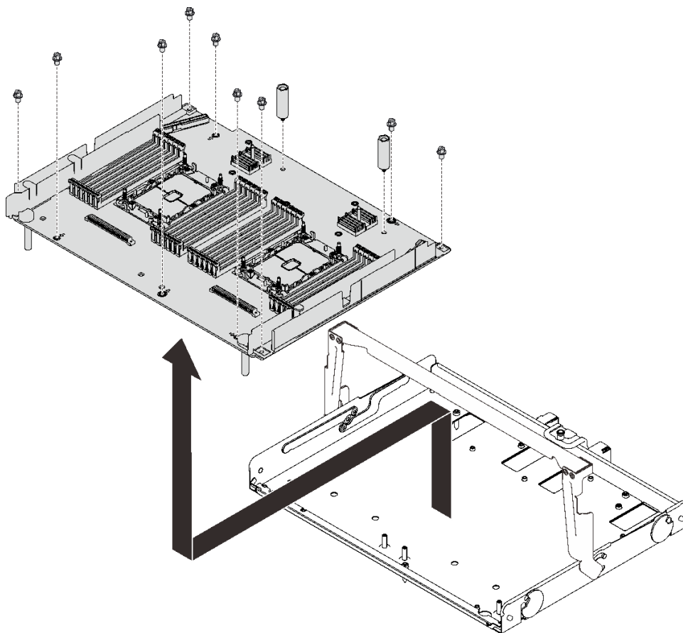
图 75. 拆卸扩展托盘
