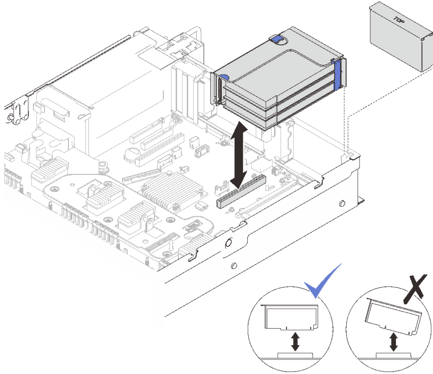
图 57. 从区域 1 中卸下 PCIe 转接卡组合件
