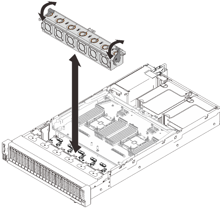
图 54. 卸下风扇架组合件
