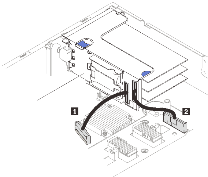
图 69. 将 PCIe 线缆从 x16/x16/x16 转接卡连接到主板
