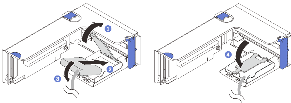
图 65. 安装快速充电模块
