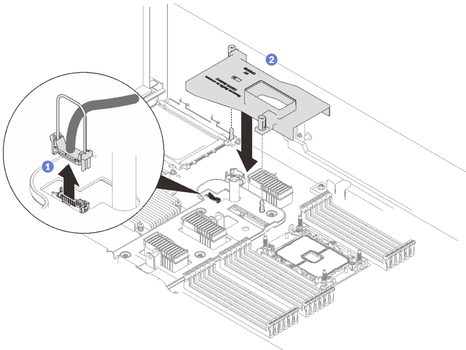
图 66. 安装 OCP 适配器导风罩
