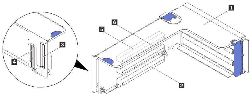
图 15. x16/x16/x16 PCIe 转接卡接口
