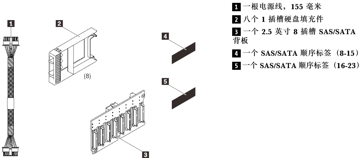
图 27. 2.5 英寸 8 插槽 SAS/SATA 背板套件
