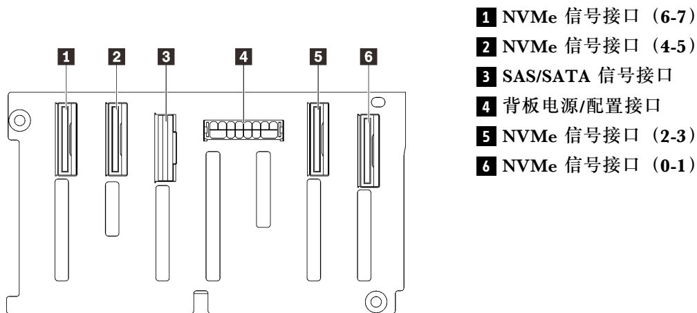
图 30. AnyBay/NVMe 硬盘背板接口
