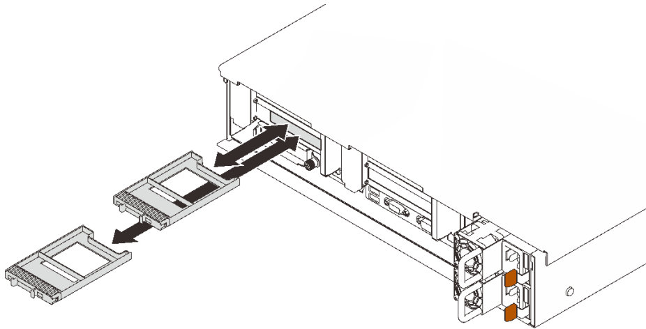
图 45. 卸下 7 毫米硬盘填充件
