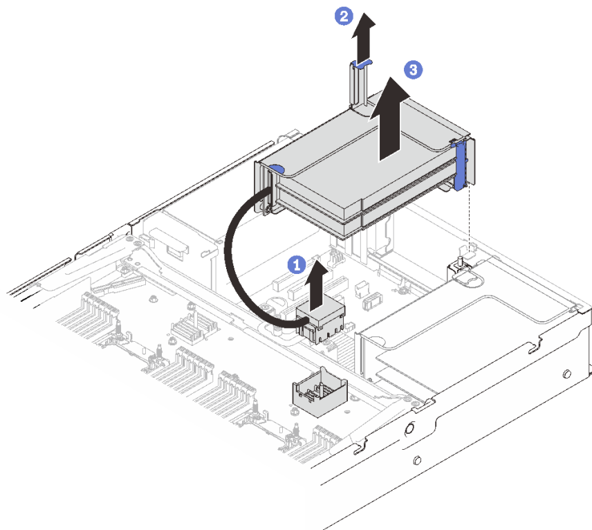
图 58. 从区域 2 中卸下 PCIe 转接卡组合件
