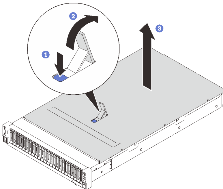
图 52. 卸下顶盖
