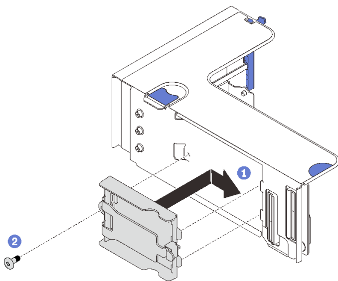
图 62. 安装垂直夹持器
