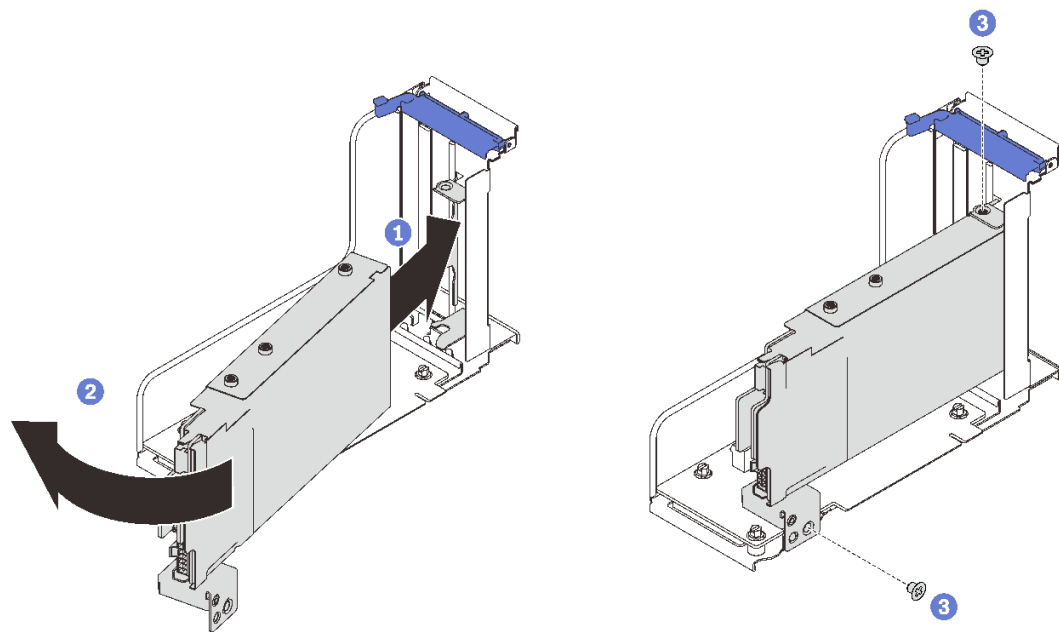
图 82. 将 7 毫米硬盘仓安装到转接卡
