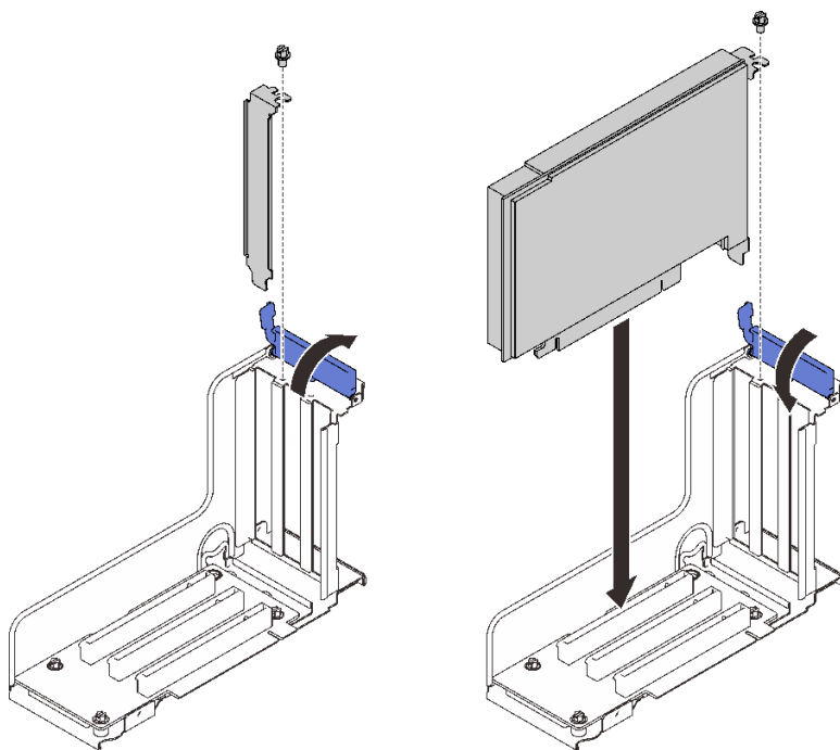
图 60. 将适配器安装到 PCIe 转接卡组合件中
