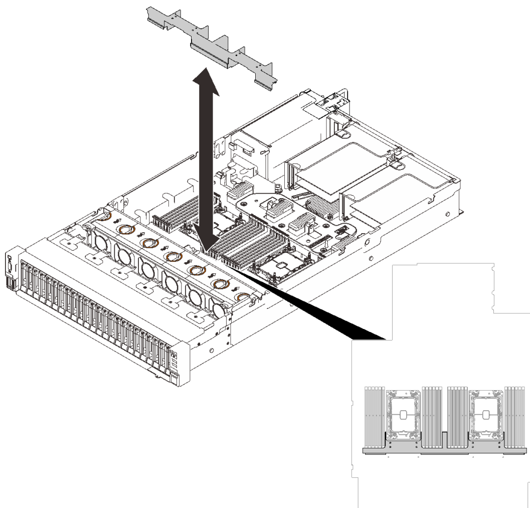
图 83. 安装扩展托盘导风罩
