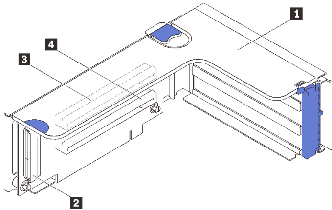
图 42. x16/x16 PCIe 转接卡接口
