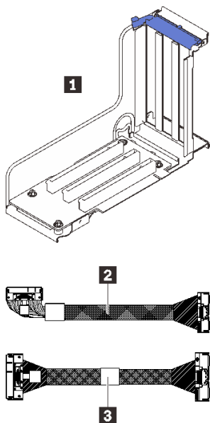
图 39. x16/x16/x16 PCIe 转接卡
