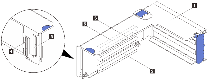
图 40. x16/x16/x16 PCIe 转接卡接口
