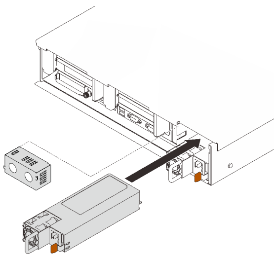
图 50. 安装电源模块单元
