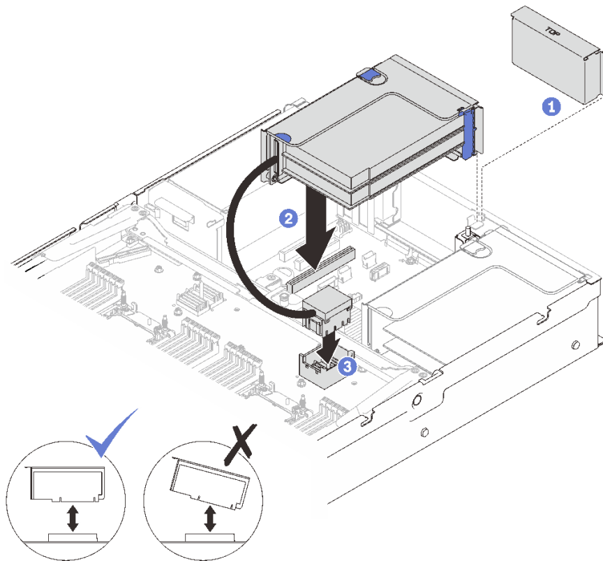
图 70. 将 PCIe 转接卡组合件安装到区域 2
