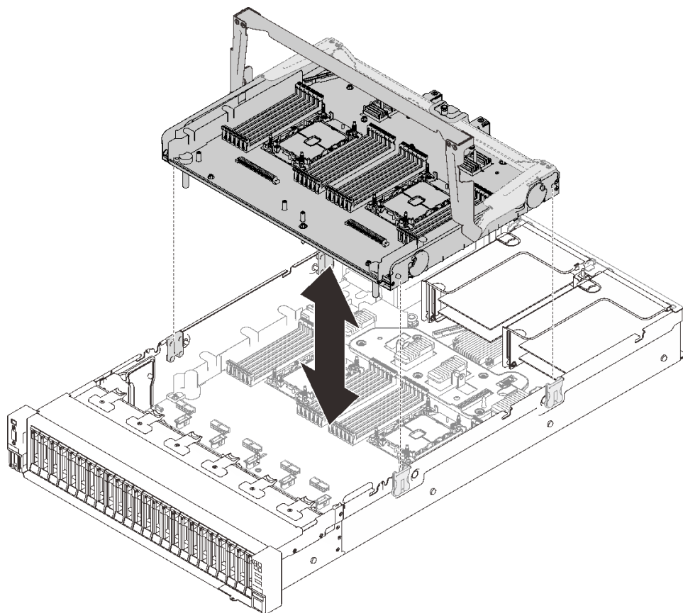
图 22. 安装处理器和内存扩展托盘
