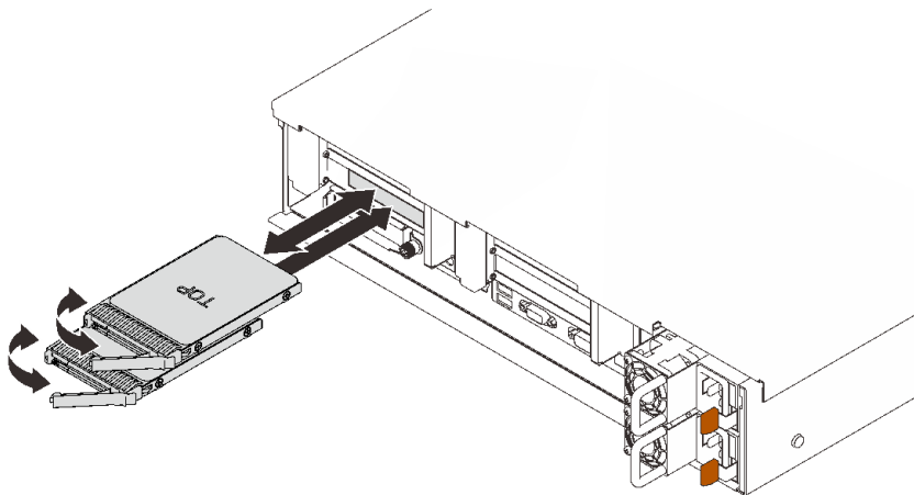
图 53. 卸下 7 毫米硬盘
