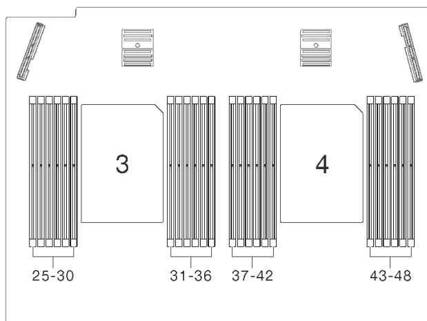
图 77. 处理器和内存扩展托盘上的处理器 3 和 4 位置
