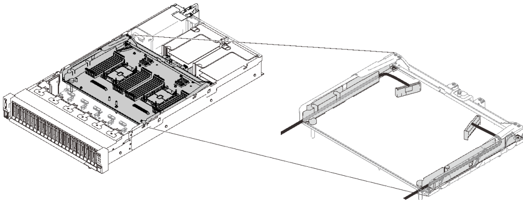
图 20. 处理器和内存扩展托盘上的线缆导轨
