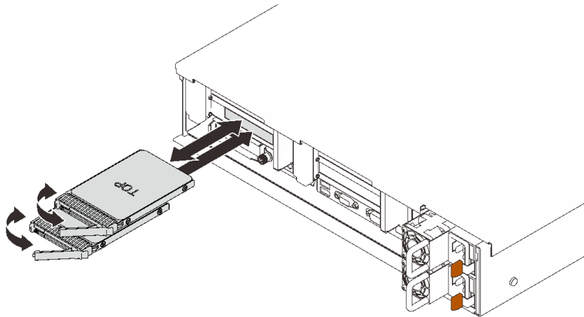
图 46. 安装 7 毫米硬盘
