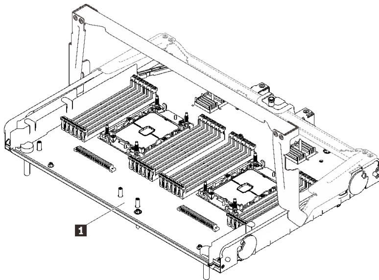
图 43. 处理器和内存扩展托盘
