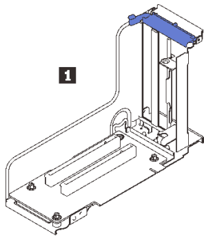
图 35. x16/x16（x8 通道）FH/HL PCIe 转接卡套件
