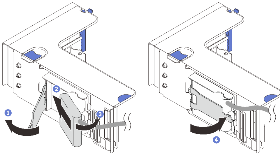
图 63. 安装快速充电模块
