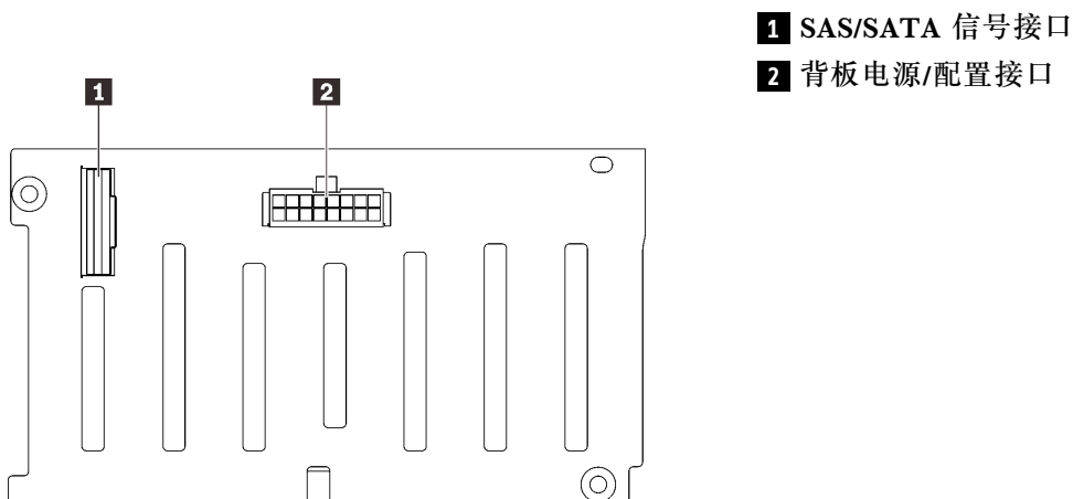
图 28. SAS/SATA 硬盘背板接口
