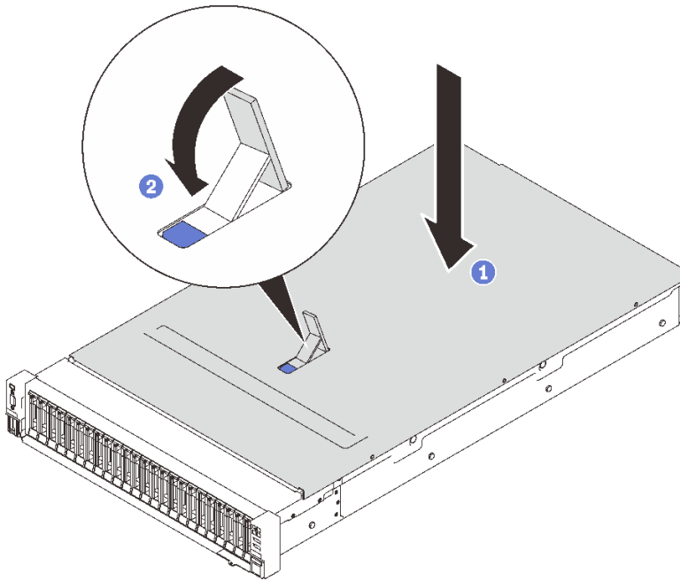
图 88. 安装顶盖
