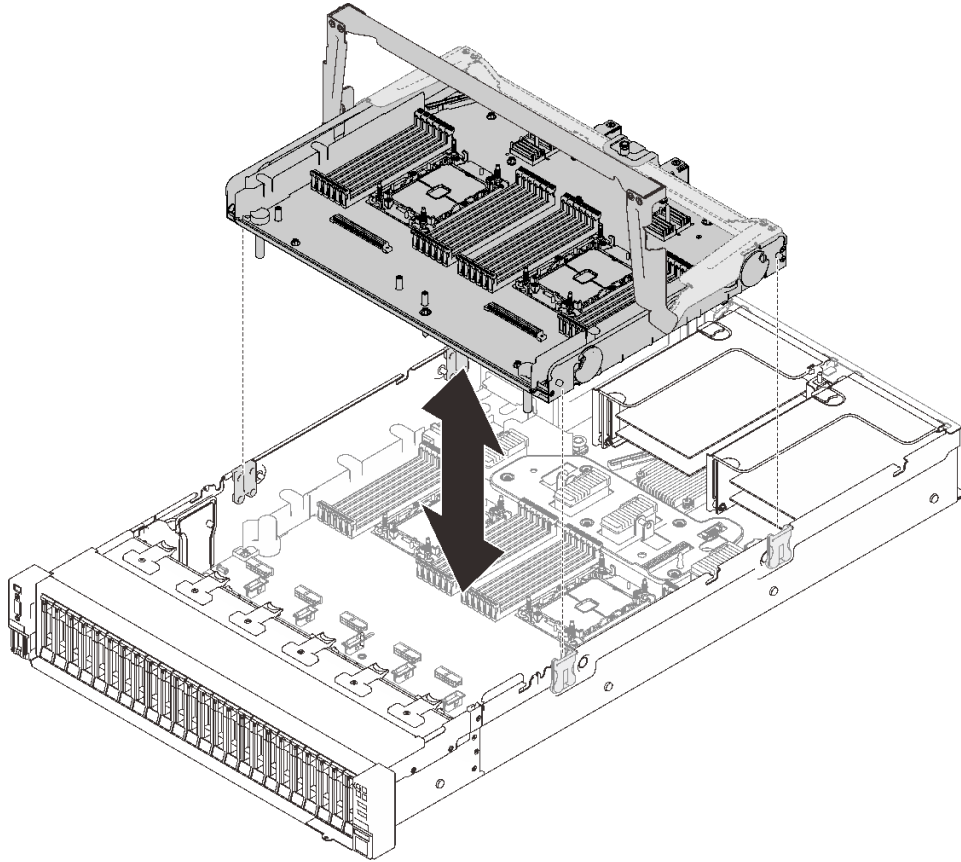
图 74. 卸下处理器和内存扩展托盘
