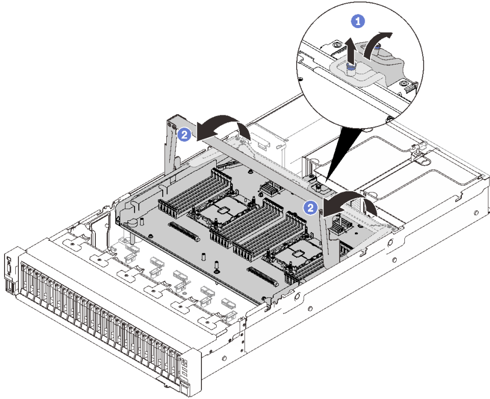
图 72. 拆卸处理器和内存扩展托盘
