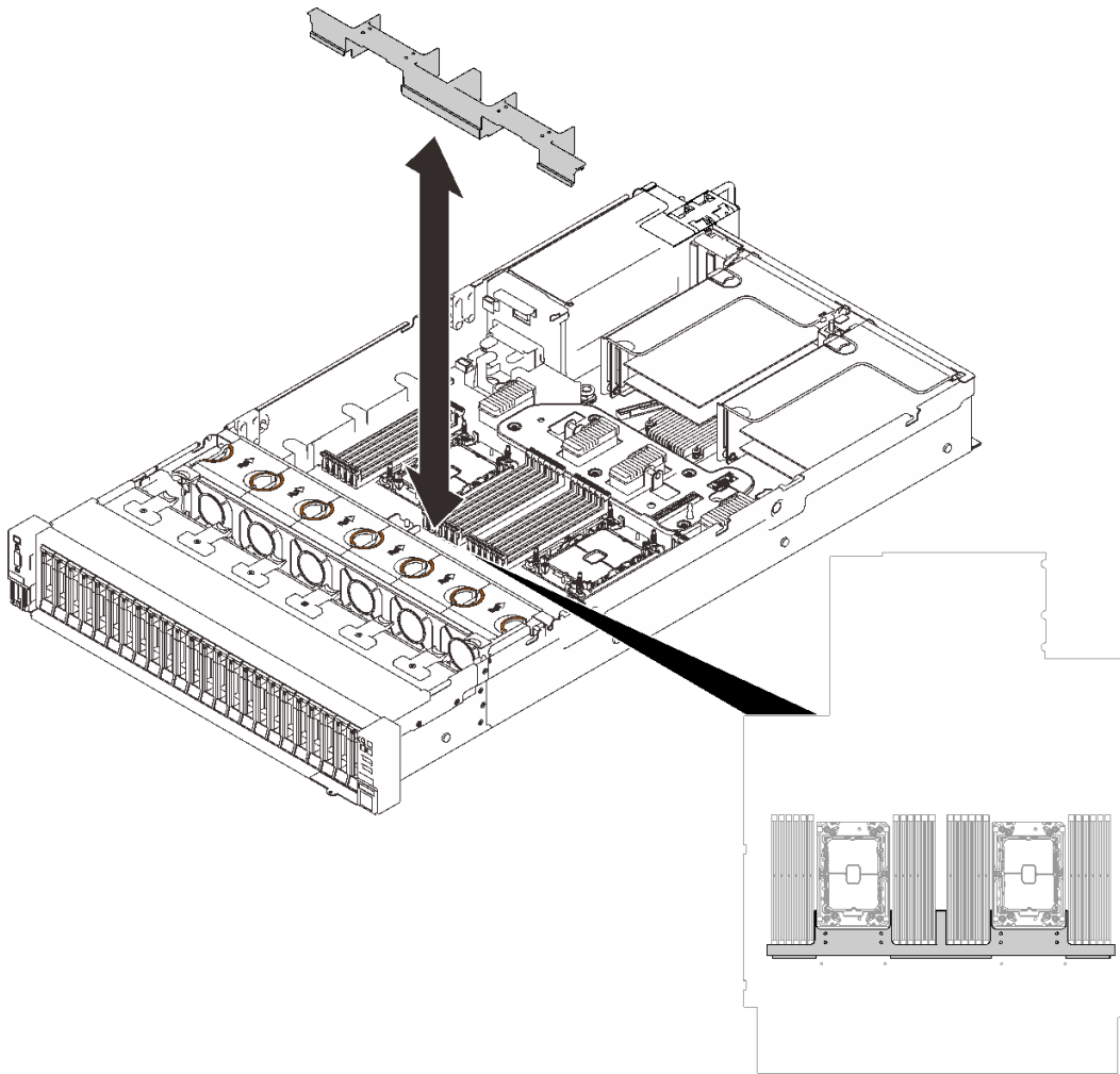
图 21. 安装扩展托盘导风罩
