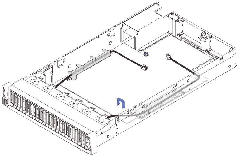
图 19. 主板上的线缆导轨
