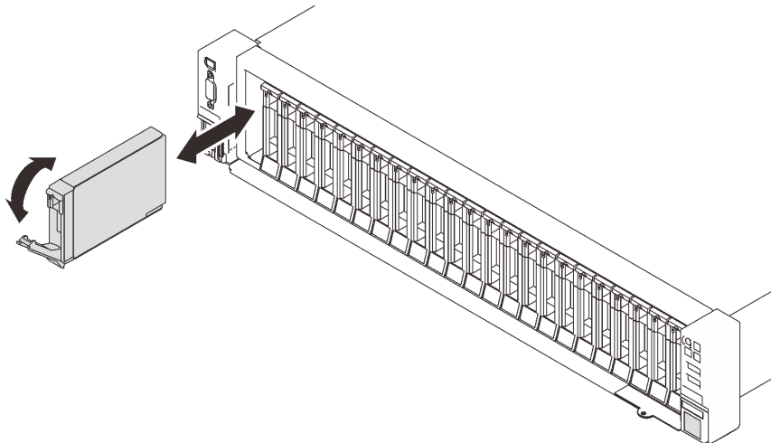
图 48. 安装 2.5 英寸硬盘
