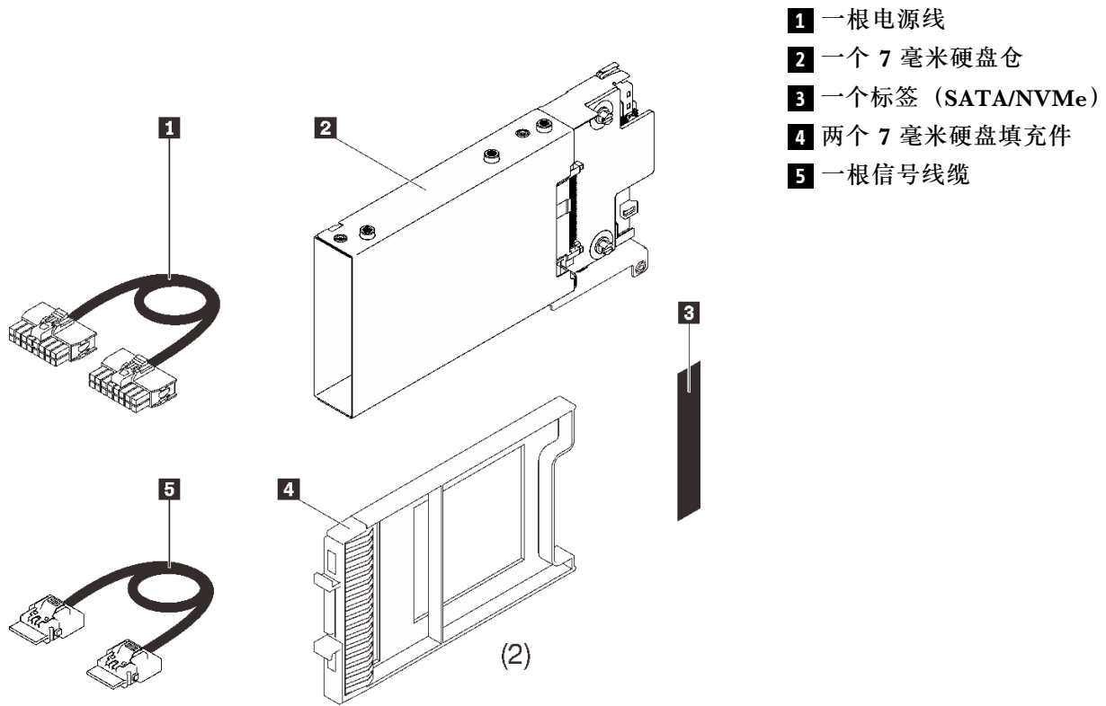
图 34. 7 毫米硬盘仓套件
