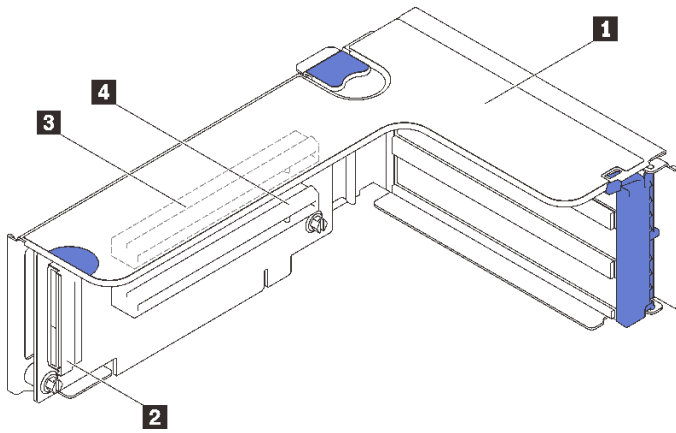
图 16. x16/x16 PCIe 转接卡接口
