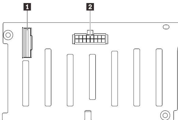
图 12. SAS/SATA 硬盘背板接口
