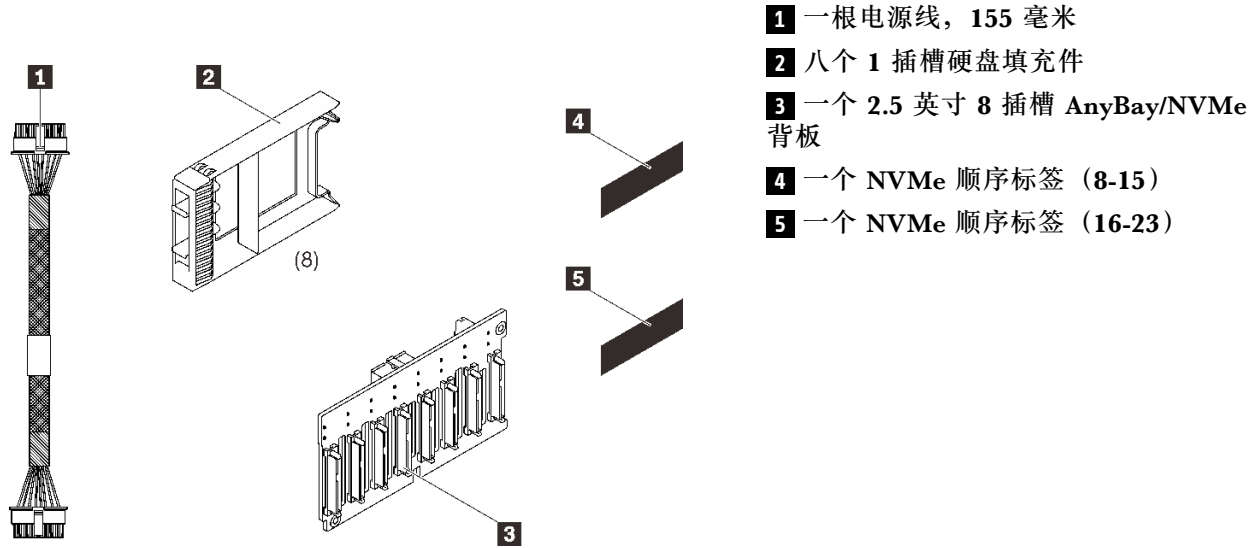
图 29. 2.5 英寸 8 插槽 SAS/SATA 背板套件
