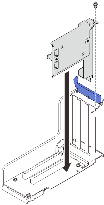
图 64. 将快速充电模块支架安装到转接卡中
