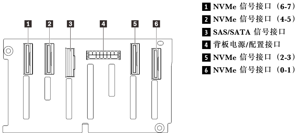
图 13. AnyBay/NVMe 硬盘背板接口
