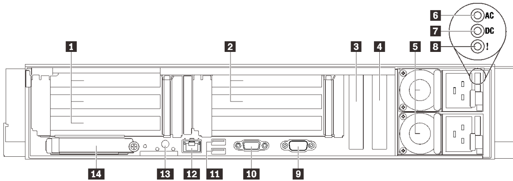
图 6. 后视图
