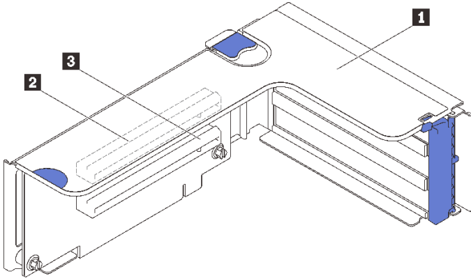
图 36. x16/x16 (x8 通道) PCIe 转接卡接口
