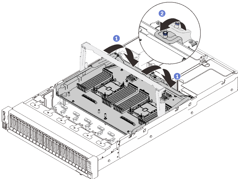
图 24. 将处理器和内存扩展托盘固定
