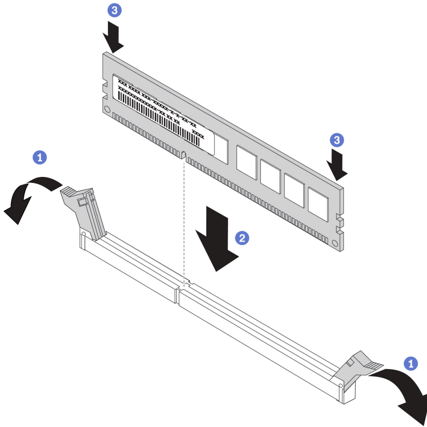
图 80. 安装内存条
