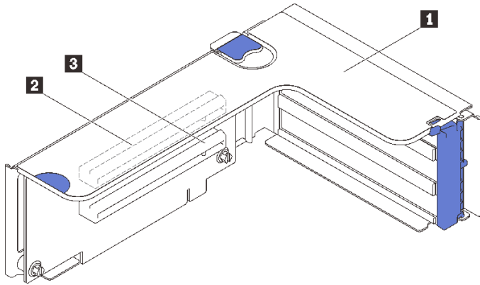
图 14. x16/x16 (x8 通道) PCIe 转接卡接口
