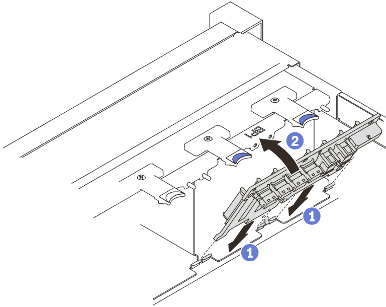
图 55. 安装硬盘背板
