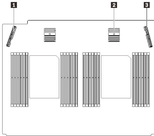
图 44. 处理器和内存扩展托盘接口
