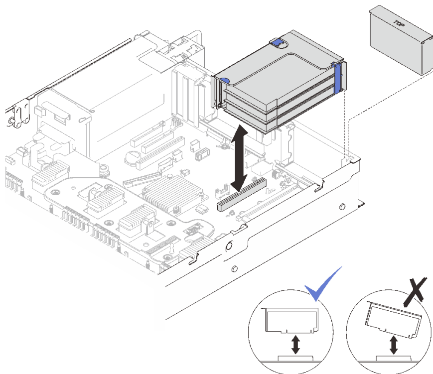
图 68. 将 PCIe 转接卡组合件安装到区域 1
