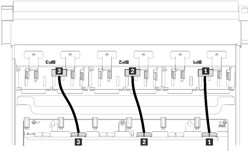
图 18. 硬盘背板电源线
