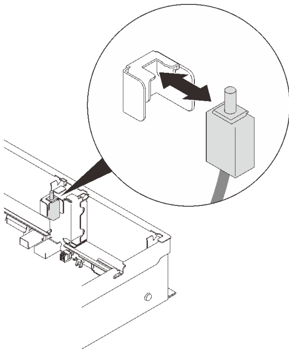
图 56. 安装入侵感应开关
