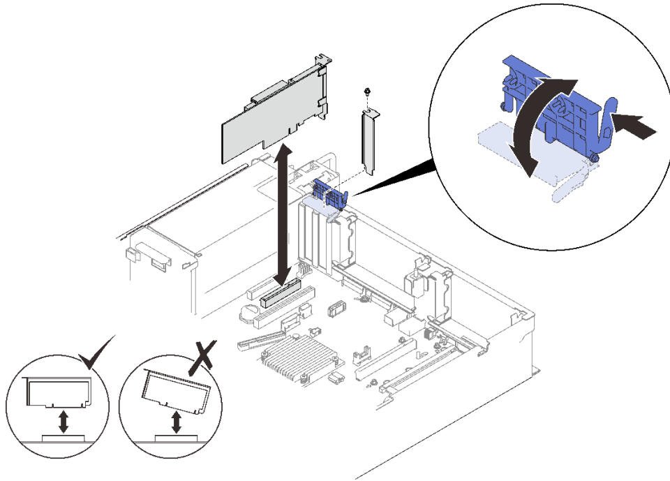
图 59. 将适配器安装到主板
