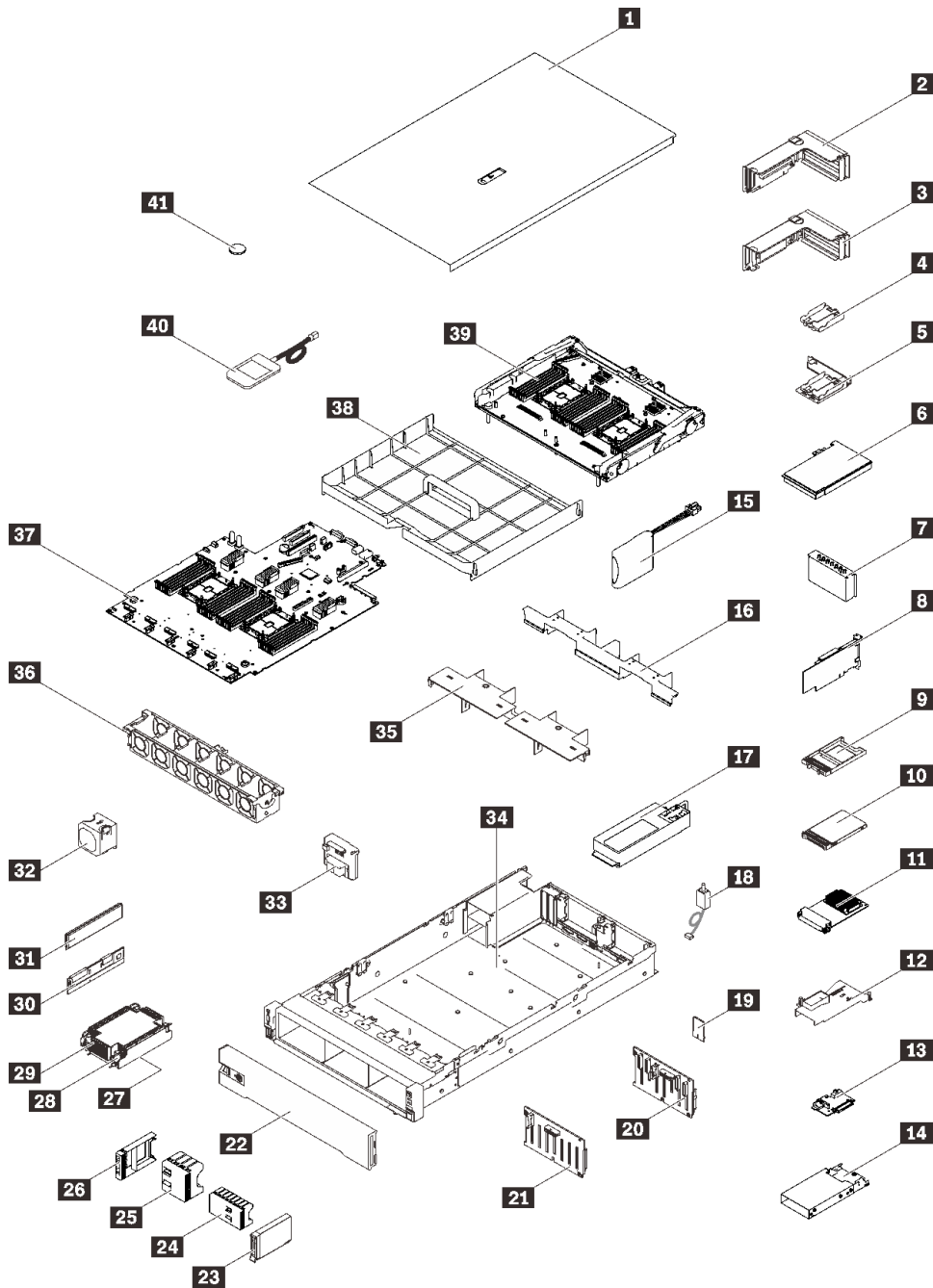
图 17. 服务器组件
