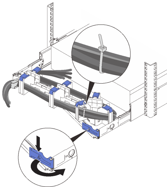
图 49. 调整 CMA
