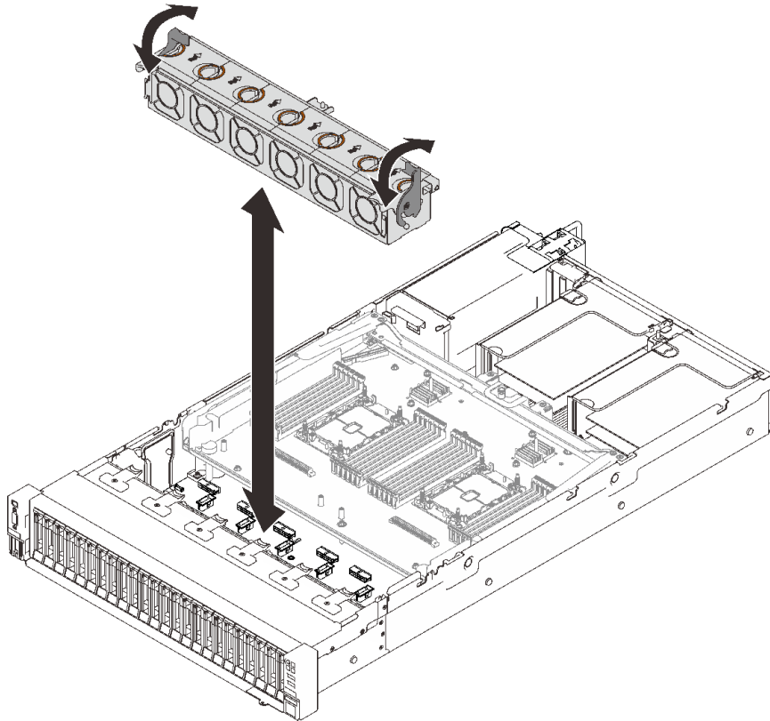
图 87. 安装风扇架组合件
