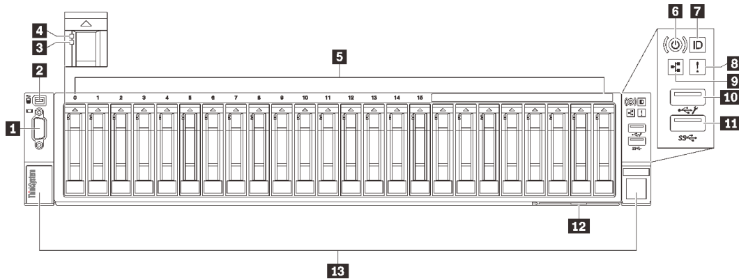
图 5. 前视图
