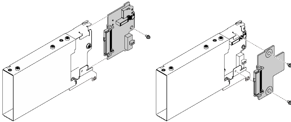
图 81. 安装 7 毫米硬盘背板
