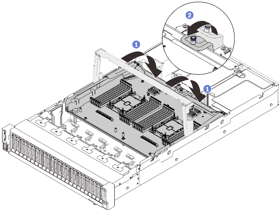
图 86. 将处理器和内存扩展托盘固定
