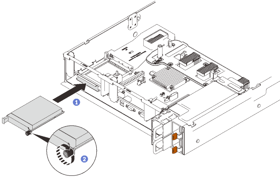
图 67. 安装 OCP 以太网适配器
