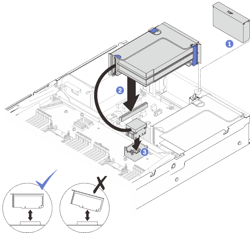
圖例 83. 將 PCIe 擴充卡組件安裝到區域 2
