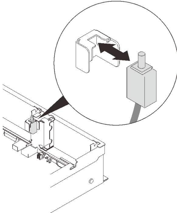
圖例 65. 安裝入侵開關
