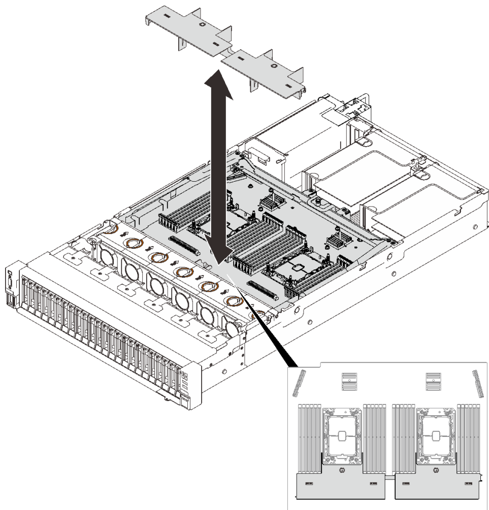
圖例 96. 從擴充匣卸下空氣擋板
