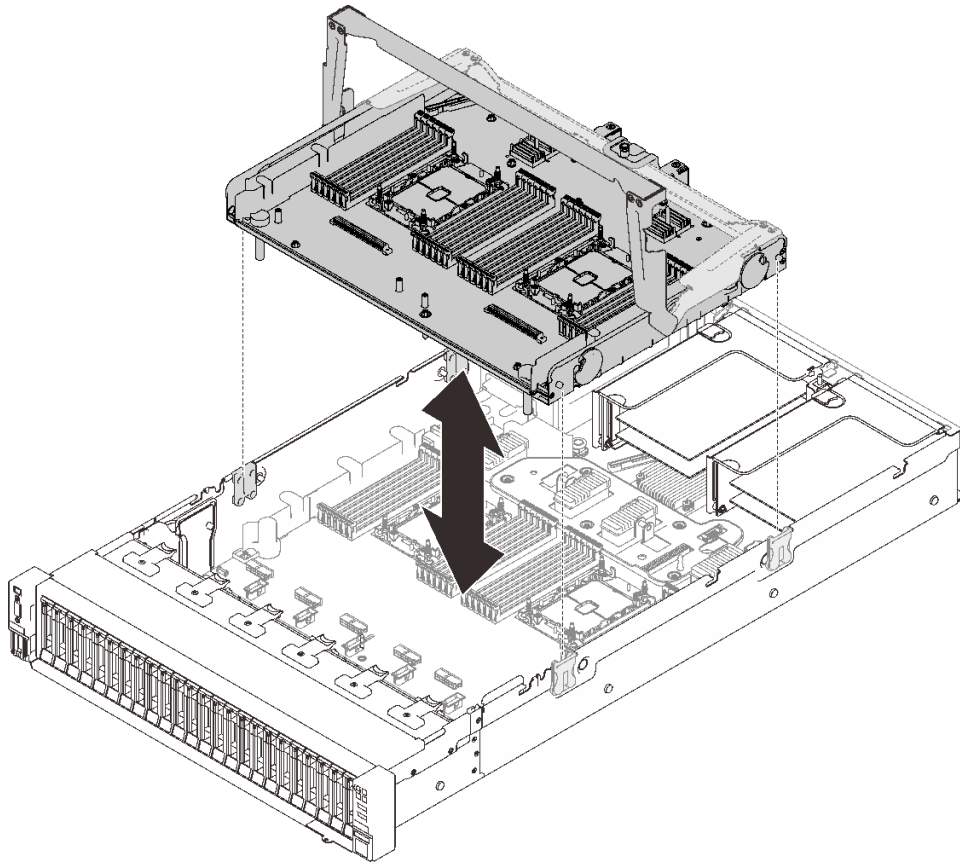
圖例 115. 安裝處理器和記憶體擴充匣
