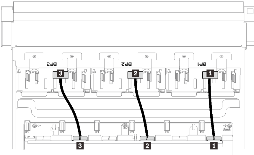
圖例 21. 硬碟背板電源線
