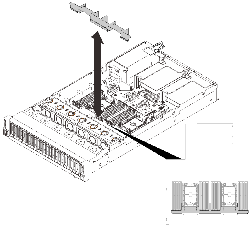
圖例 69. 卸下擴充匣空氣擋板。
