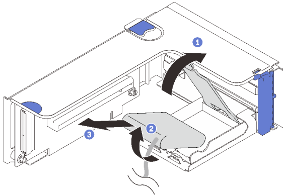
圖例 53. 從垂直固定器卸下快閃記憶體電源模組
