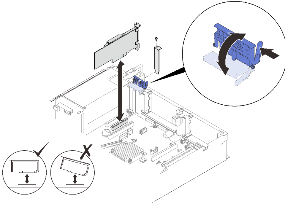
圖例 79. 將配接卡安裝到主機板
