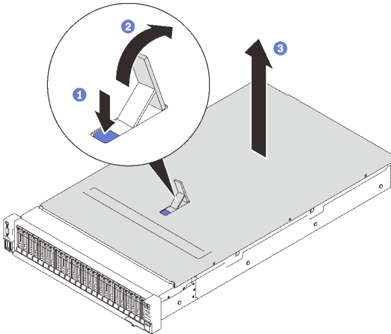
圖例 130. 卸下上蓋
