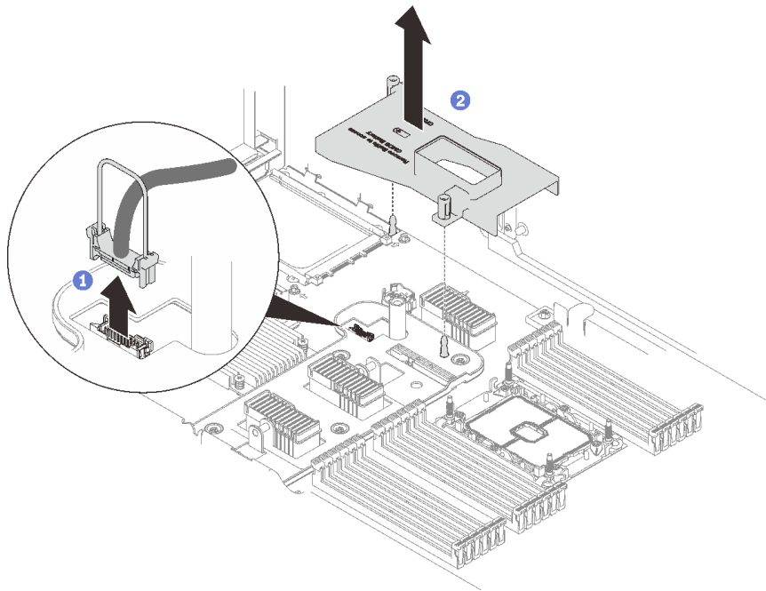
圖例 42. 卸下 OCP 配接卡空氣擋板
