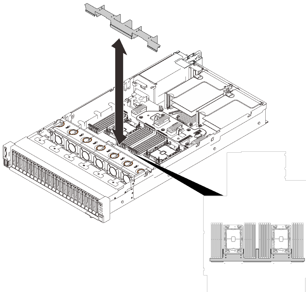
圖例 133. 將空氣擋板安裝到主機板
