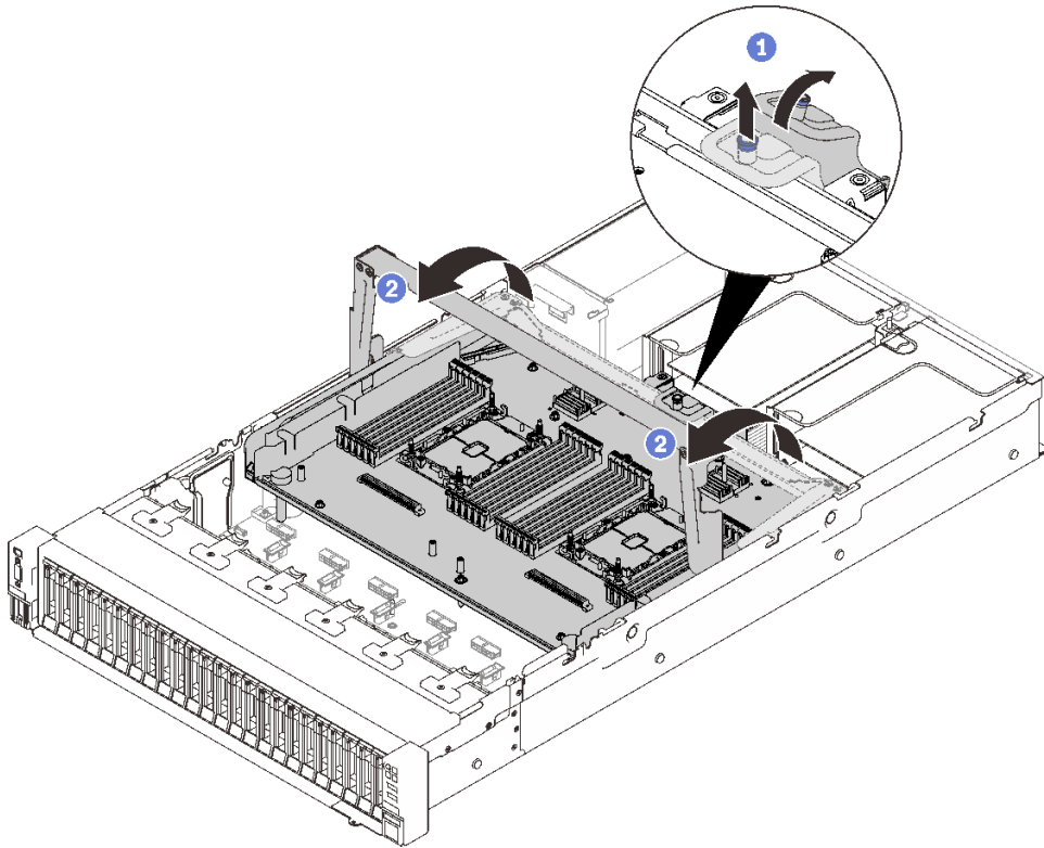
圖例 110. 鬆開處理器和記憶體擴充匣
