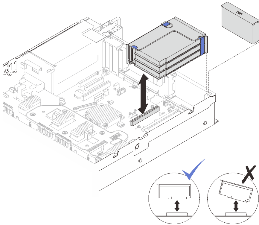
圖例 74. 從區域 1 卸下 PCIe 擴充卡組件
