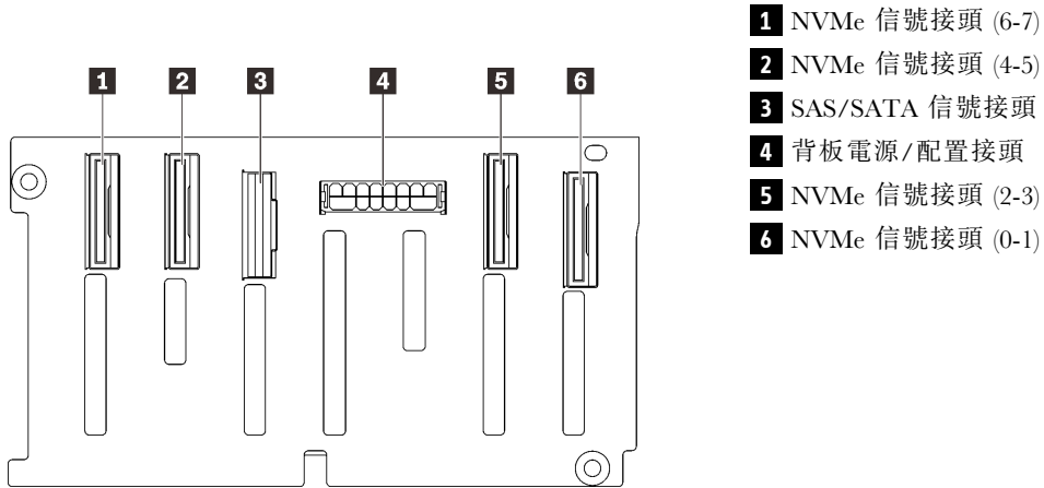
圖例 13. AnyBay/NVMe 硬碟背板接頭
