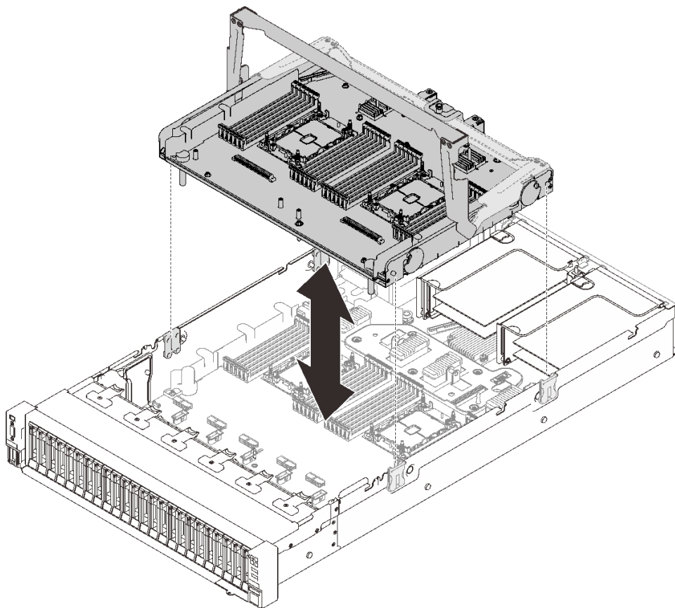
圖例 112. 卸下處理器和記憶體擴充匣
