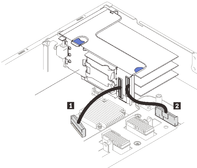
圖例 82. 將 PCIe 纜線從 x16/x16/x16 擴充卡連接到主機板
