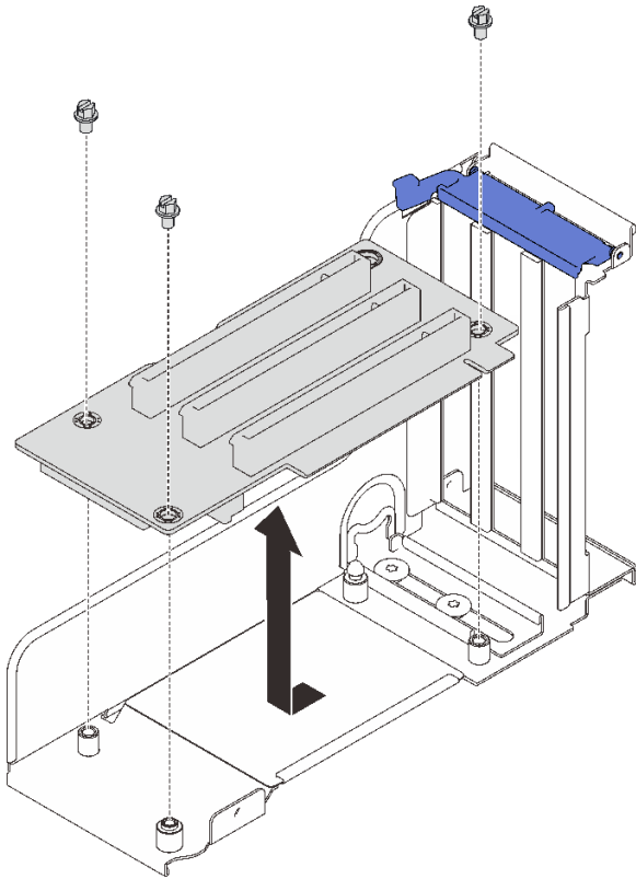
圖例 76. 拆卸 PCIe 擴充卡
