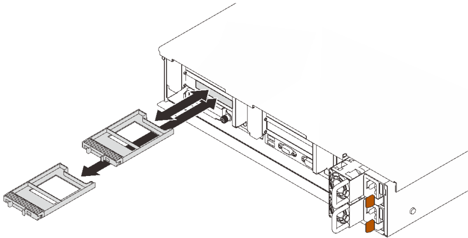
圖例 40. 卸下 7 公釐硬碟填充板
