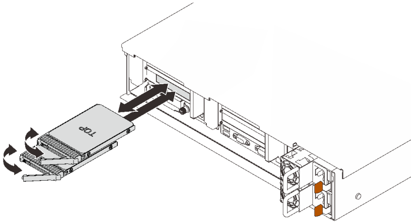
圖例 34. 卸下 7 公釐硬碟
