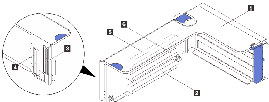
圖例 15. x16/x16/x16 PCIe 擴充卡接頭
