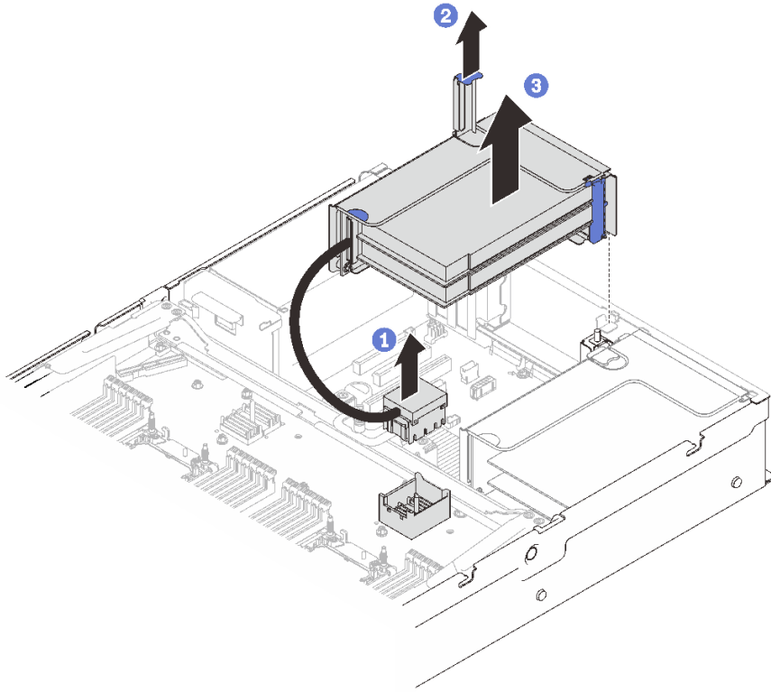
圖例 75. 從區域 2 卸下 PCIe 擴充卡組件
