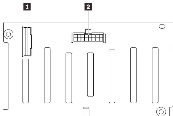
圖例 12. SAS/SATA 硬碟背板接頭
