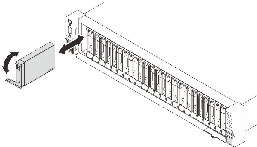
圖例 29. 卸下 2.5 吋硬碟
