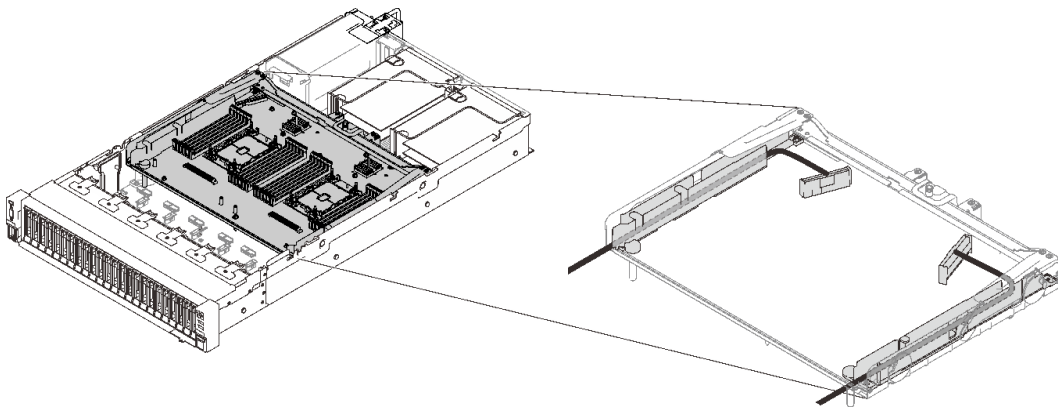
圖例 23. 處理器和記憶體擴充匣上的纜線導件
