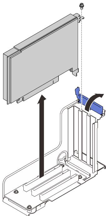
圖例 78. 從 PCIe 擴充卡組件卸下配接卡
