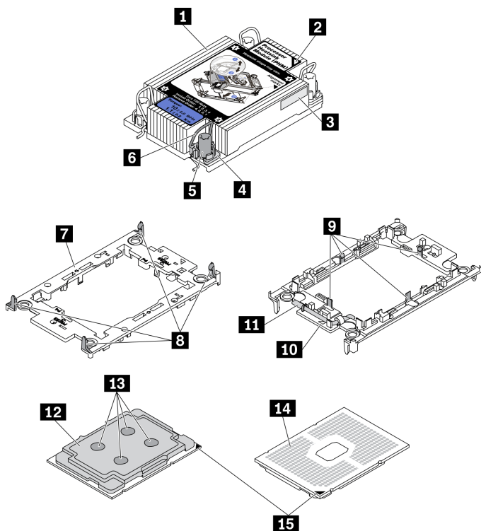
圖例 104. PHM 元件
