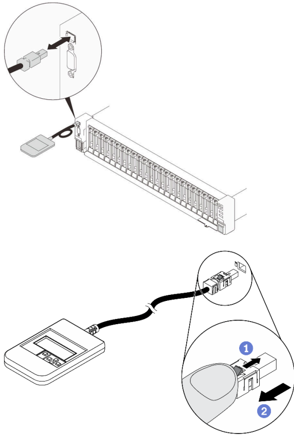
圖例 46. 拔掉外部 LCD 診斷手持裝置纜線
