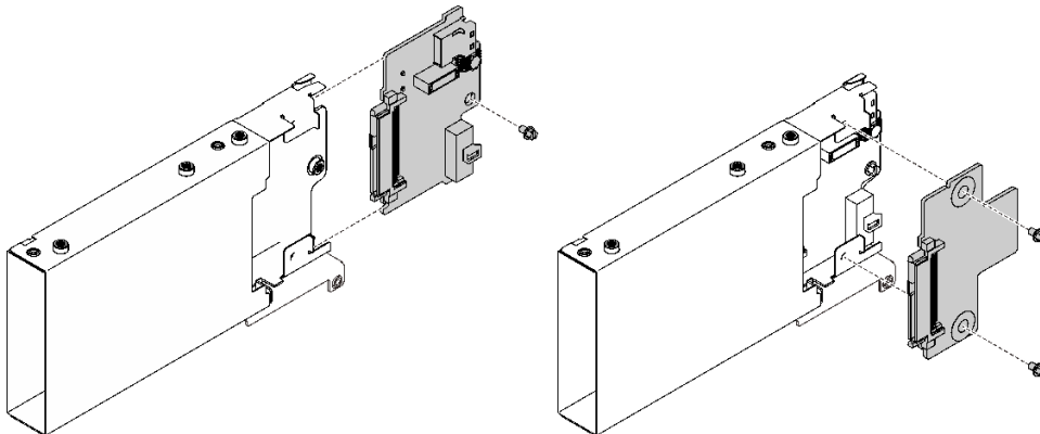
圖例 38. 安裝 7 公釐硬碟背板
