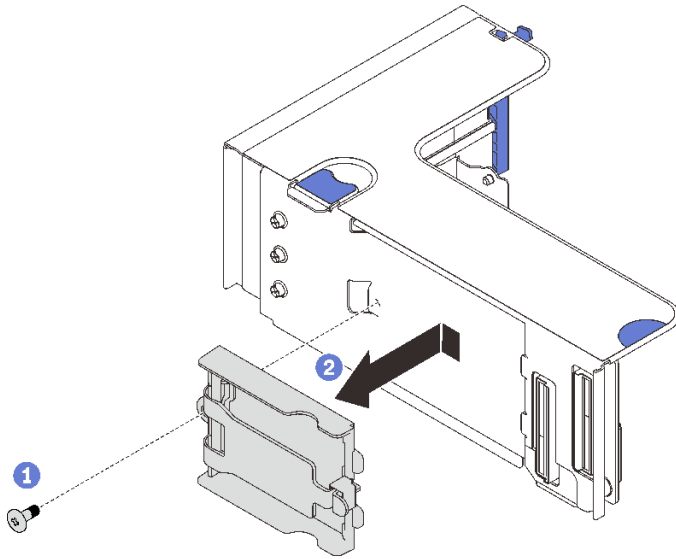
圖例 55. 卸下垂直固定器
