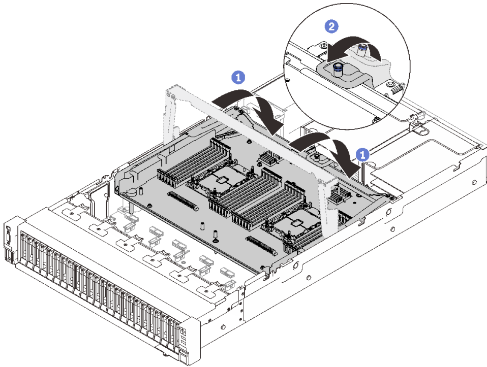
圖例 27. 固定處理器和記憶體擴充匣
