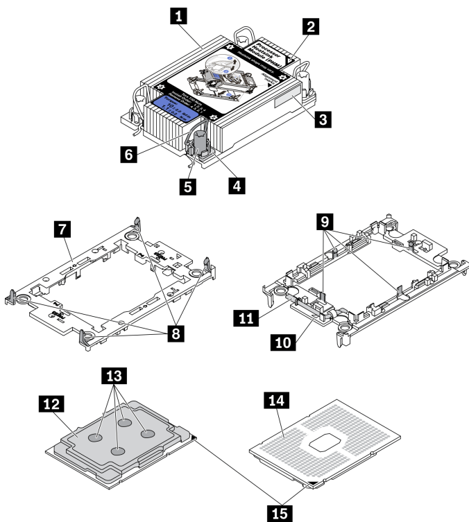
圖例 95. PHM 元件
