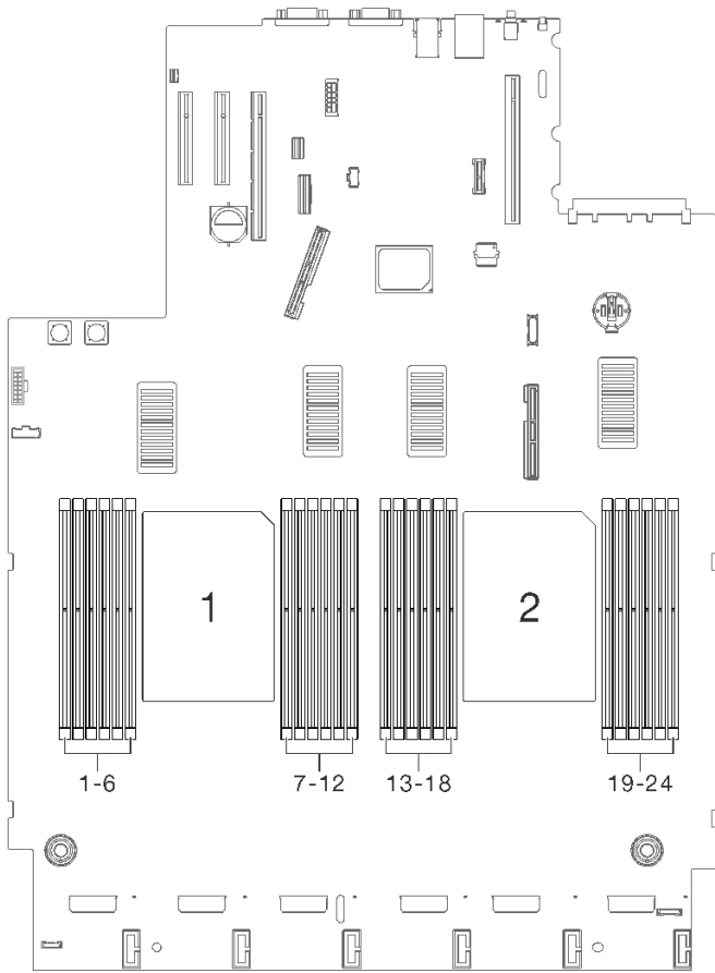
圖例 66. 主機板上的記憶體模組插槽 1-24
