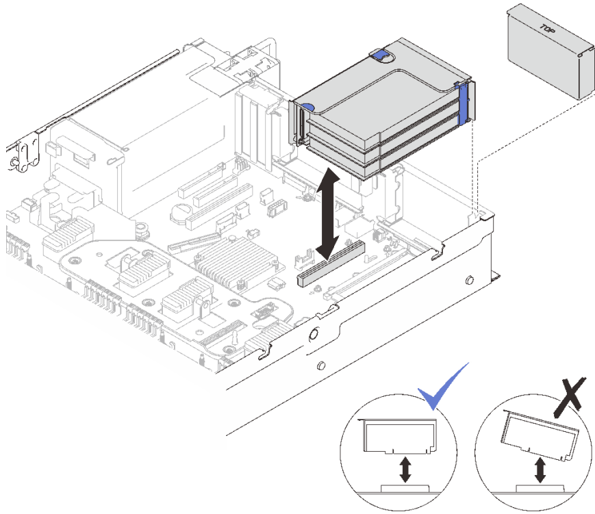
圖例 81. 將 PCIe 擴充卡組件安裝到區域 1
