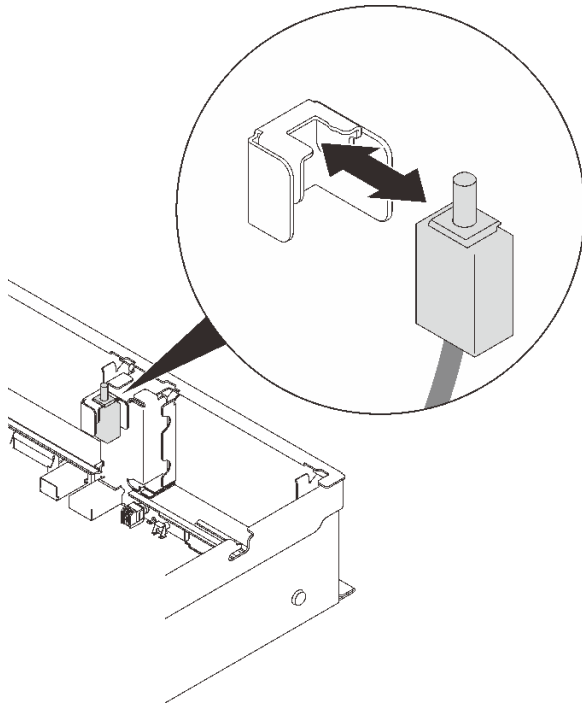
圖例 64. 卸下入侵開關
