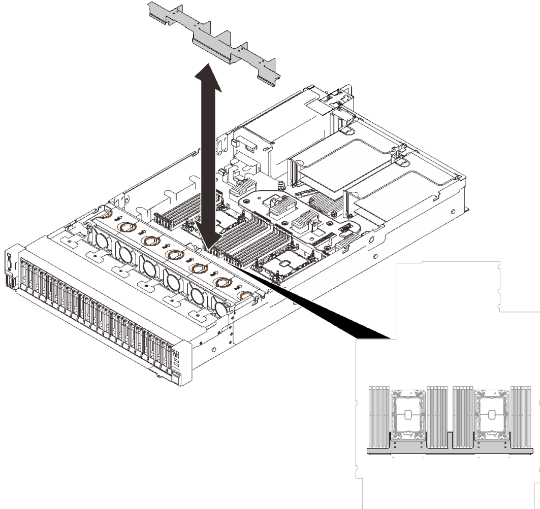
圖例 97. 卸下擴充匣空氣擋板。
