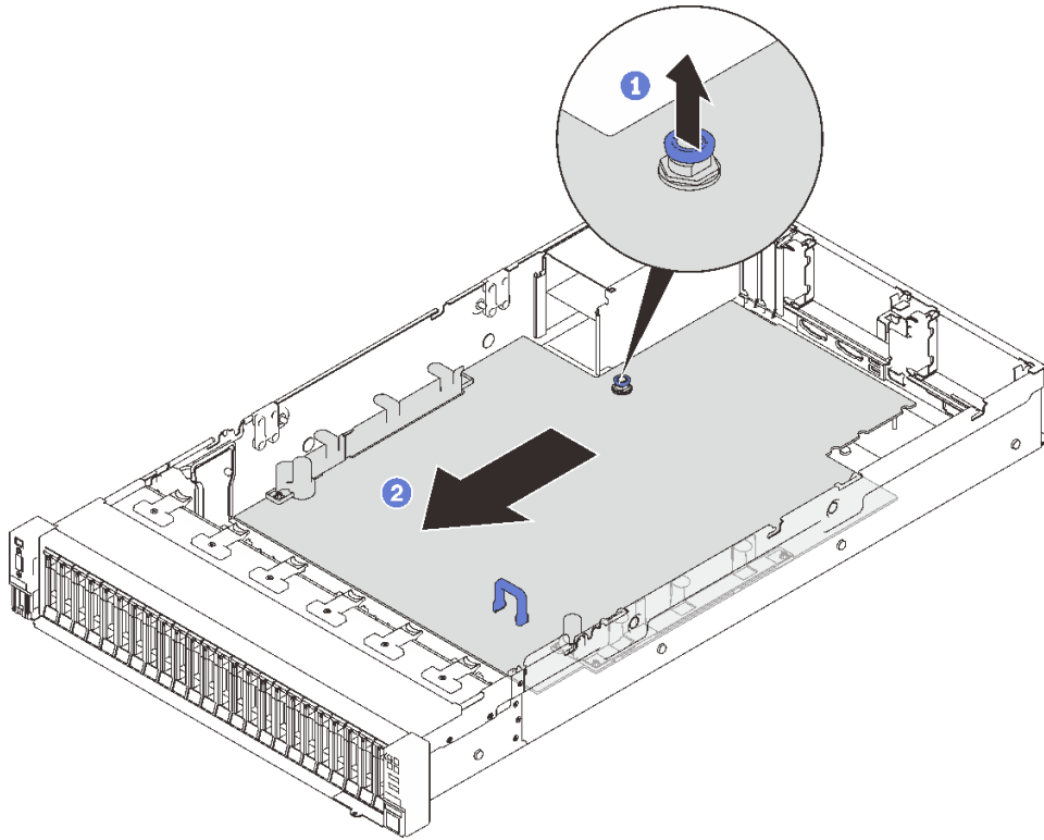
圖例 124. 鬆開主機板
