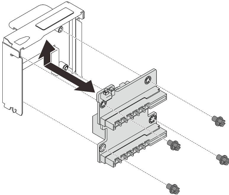
圖例 86. 拆卸電源背板
