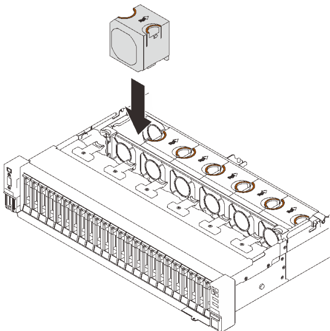
圖例 52. 安裝風扇
