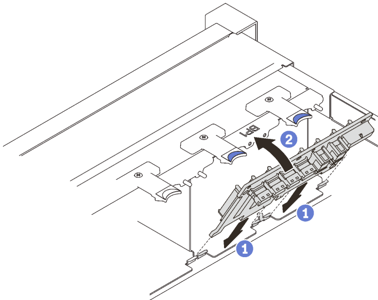
圖例 31. 安裝硬碟背板
