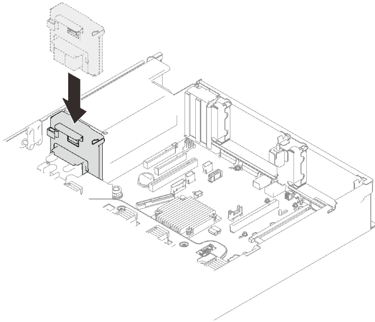
圖例 87. 安裝電源背板
