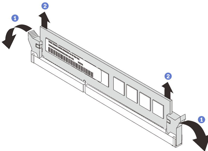
圖例 70. 卸下記憶體模組
