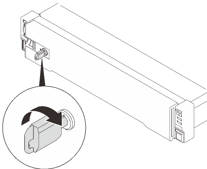
圖例 118. 解鎖安全擋板
