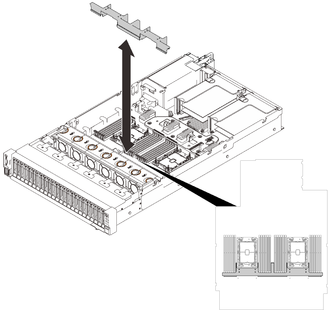
圖例 61. 卸下擴充匣空氣擋板。
