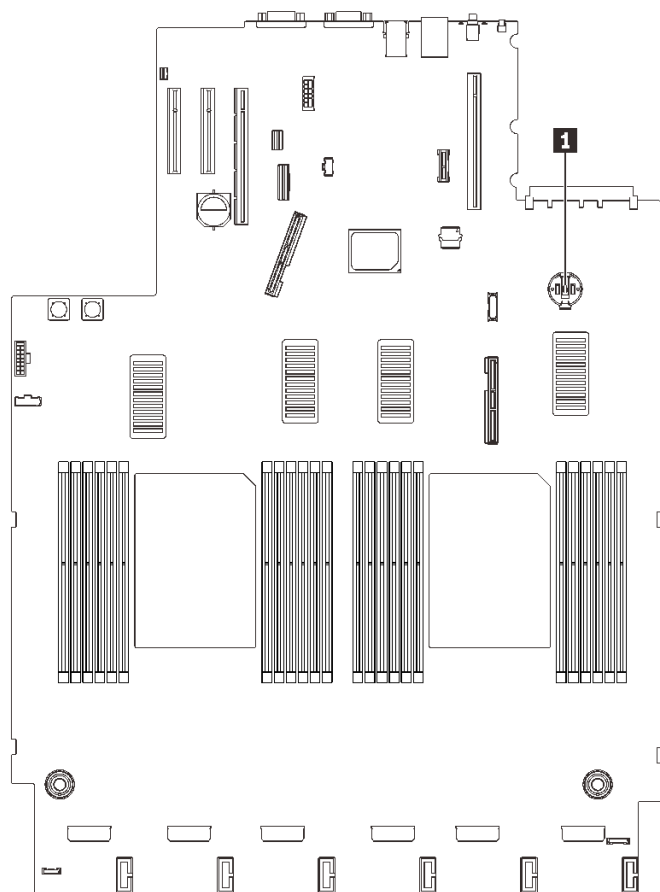
圖例 43. 主機板上的 CMOS 電池位置
