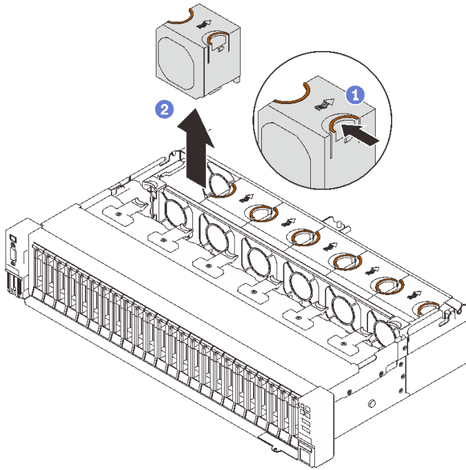
圖例 51. 卸下風扇
