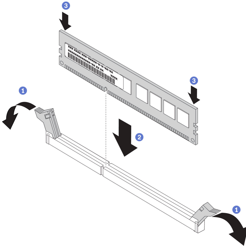
圖例 71. 安裝記憶體模組
