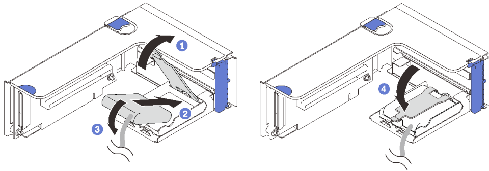
圖例 58. 將快閃記憶體電源模組安裝到水平固定器中
