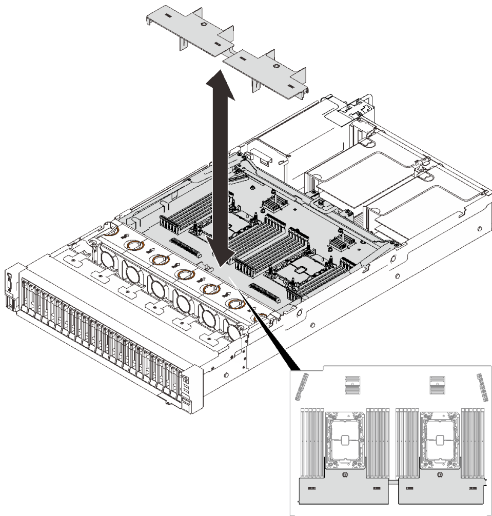
圖例 68. 從擴充匣卸下空氣擋板
