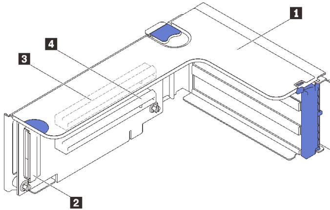
圖例 16. x16/x16 PCIe 擴充卡接頭
