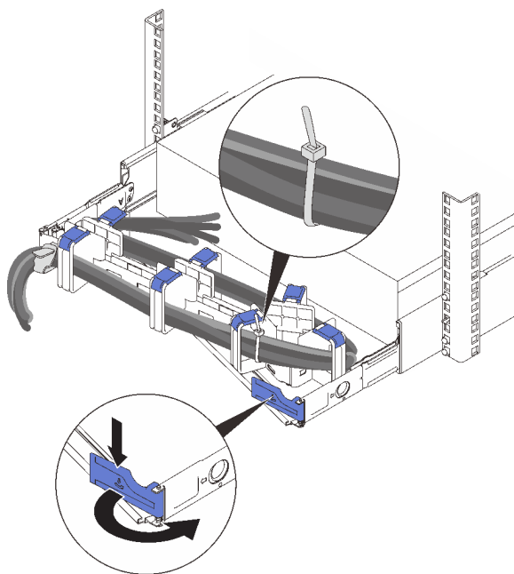
圖例 91. 調整 CMA
