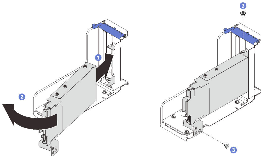
圖例 39. 將 7 公釐框架安裝到擴充卡
