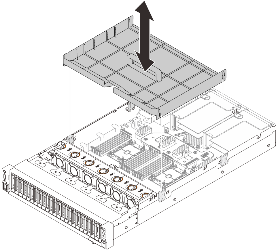
圖例 123. 安裝主機板空氣擋板
