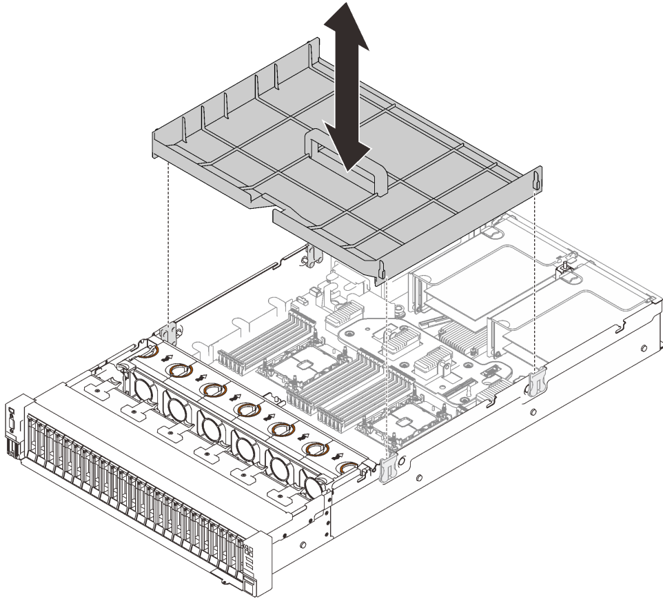
圖例 122. 卸下主機板空氣擋板
