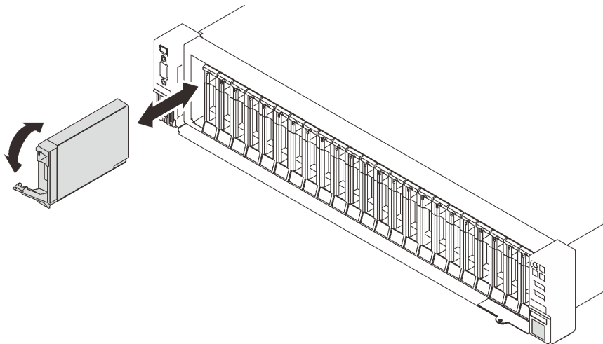
圖例 33. 安裝 2.5 吋硬碟
