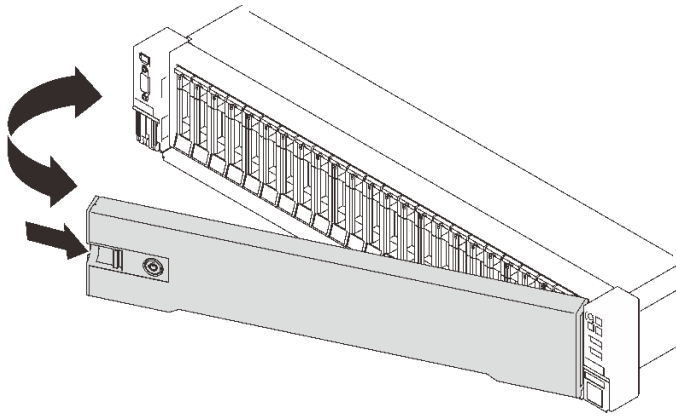
圖例 119. 卸下安全擋板
