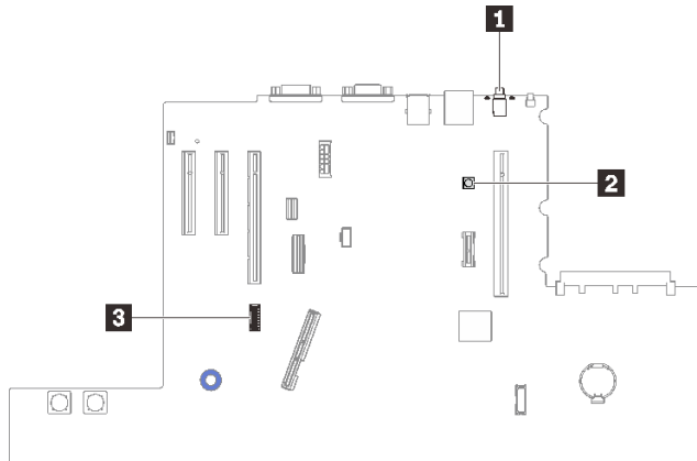
圖例 17. 開關、跳接器和按鈕
