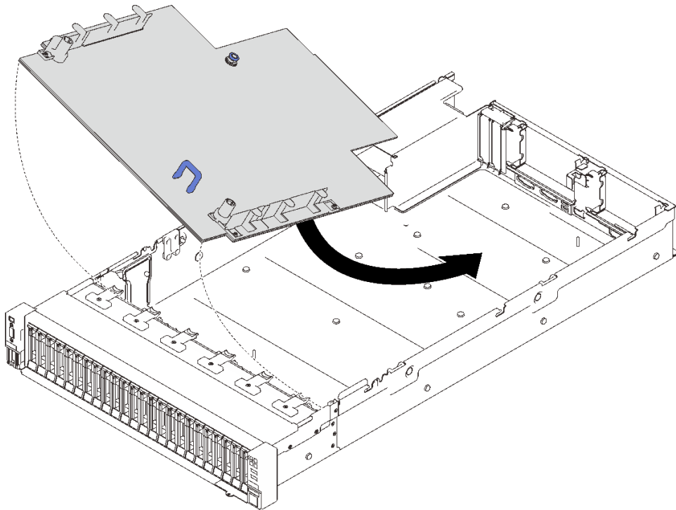
圖例 127. 安裝主機板
