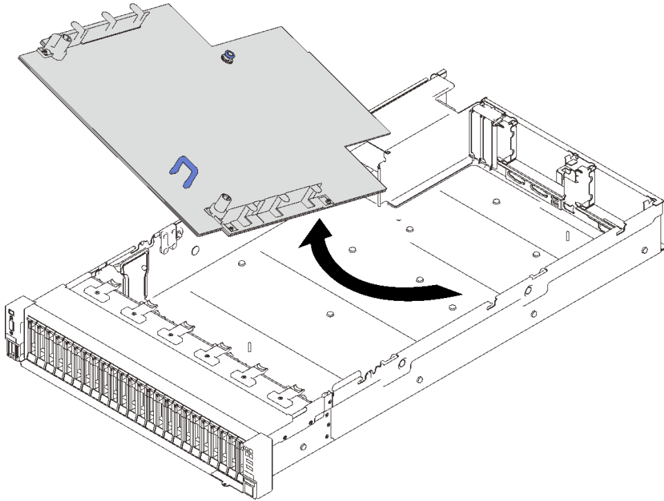
圖例 125. 卸下主機板
