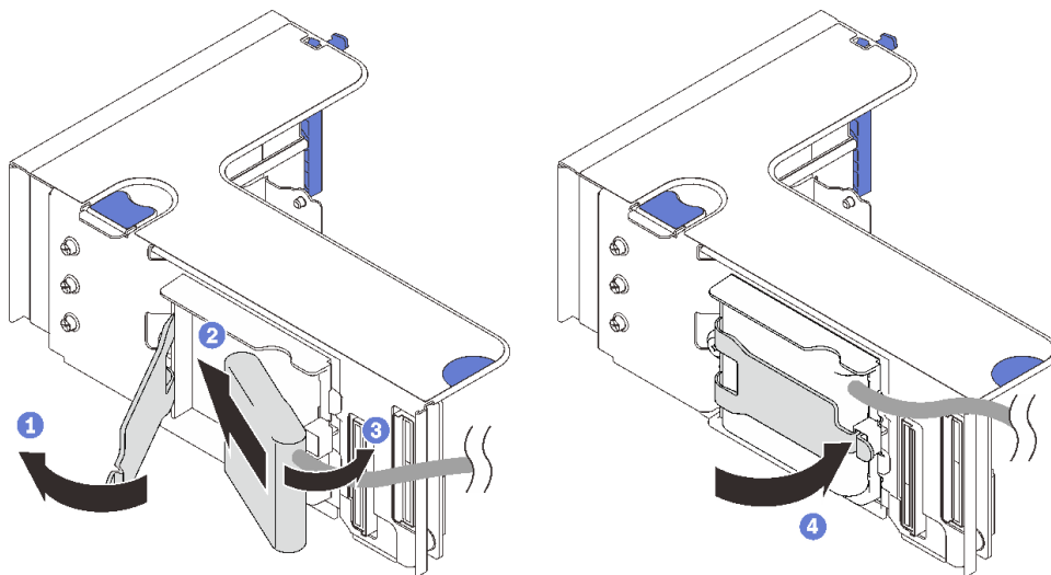
圖例 59. 將快閃記憶體電源模組安裝到垂直固定器中
