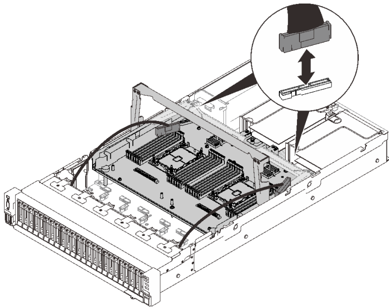
圖例 111. 拔掉 PCIe 纜線
