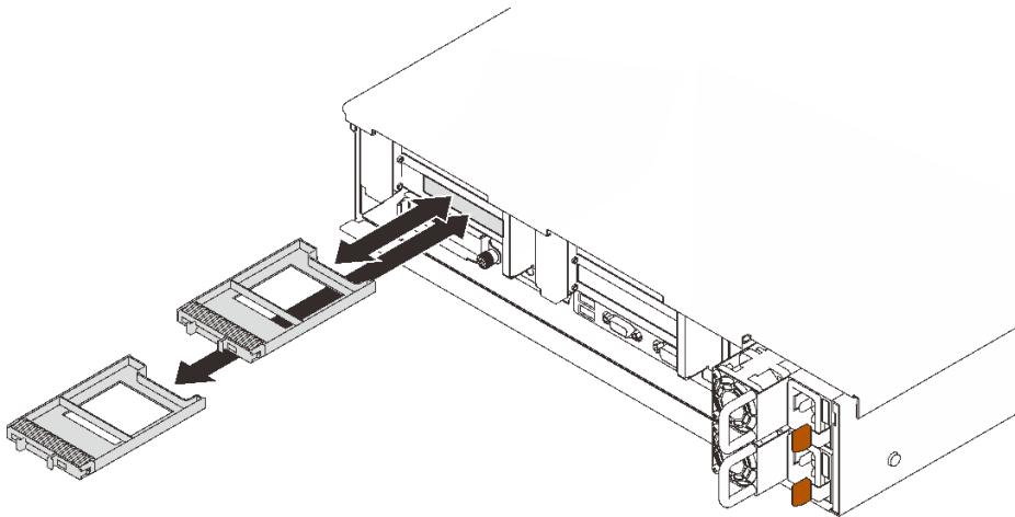
圖例 35. 安裝 7 公釐硬碟填充板
