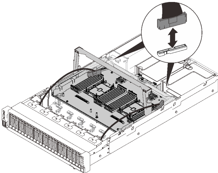
圖例 26. 將纜線連接到擴充匣
