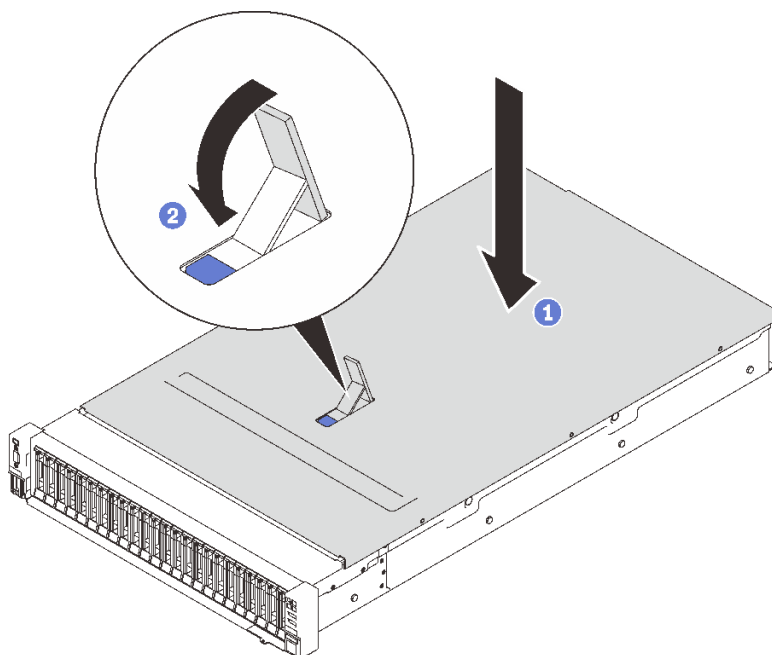
圖例 131. 安裝上蓋
