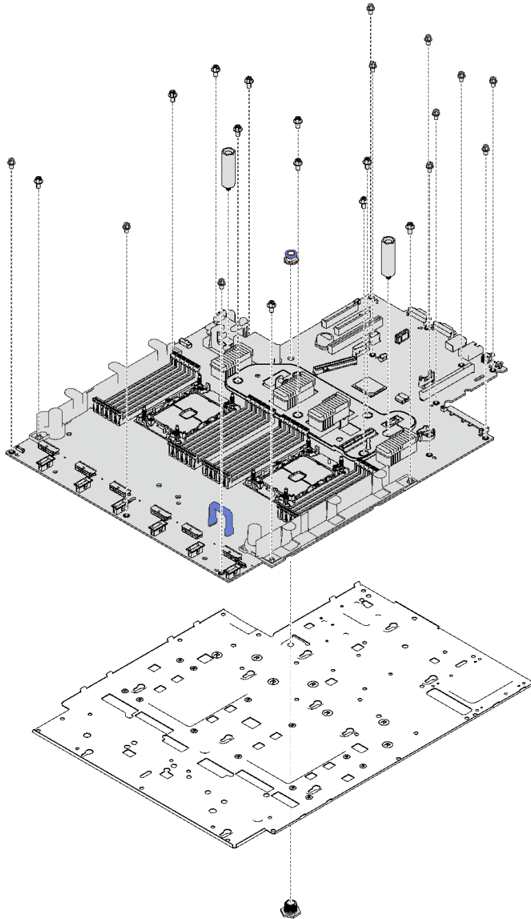
圖例 126. 拆卸主機板
