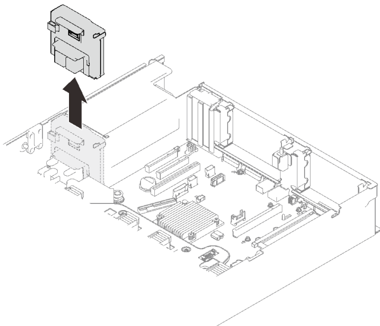
圖例 85. 卸下電源背板
