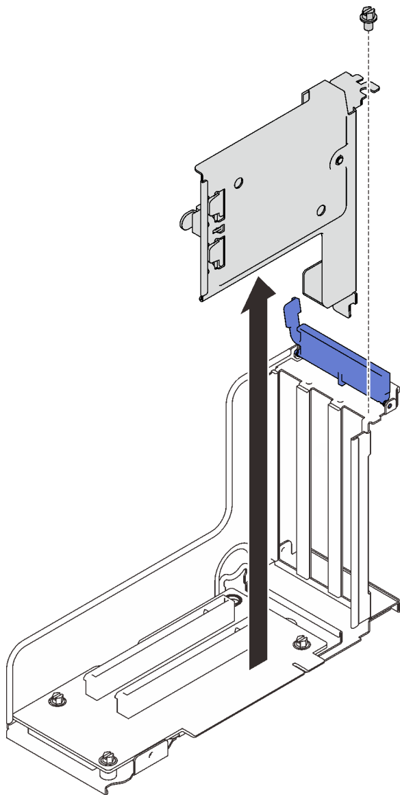
圖例 56. 從 PCIe 擴充卡卸下匣托架
