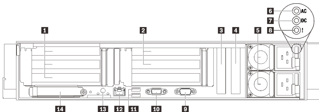
圖例 6. 背面圖
