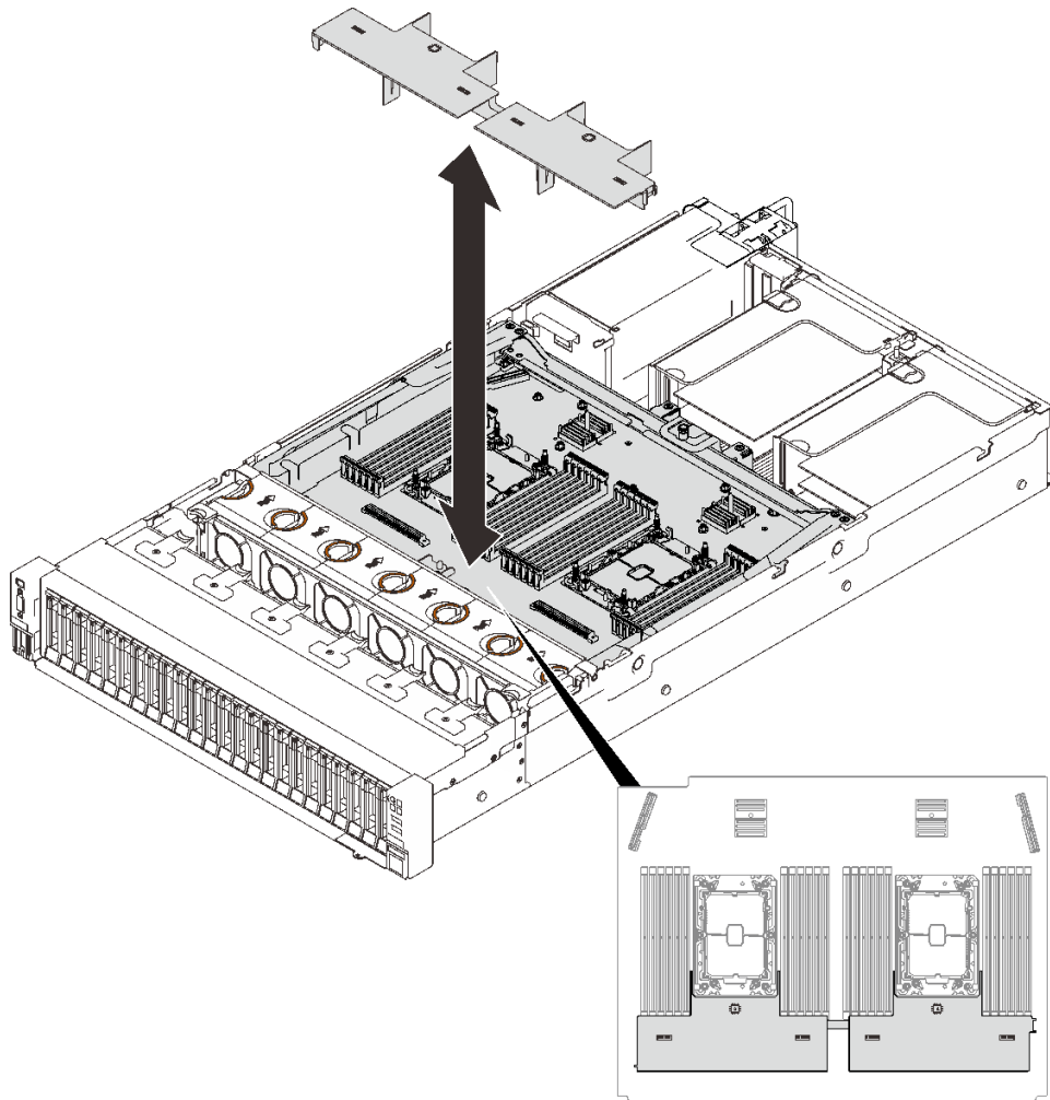
圖例 134. 將空氣擋板安裝到擴充匣
