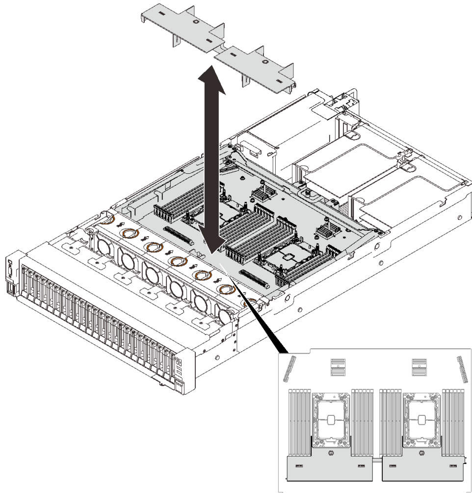
圖例 60. 從擴充匣卸下空氣擋板
