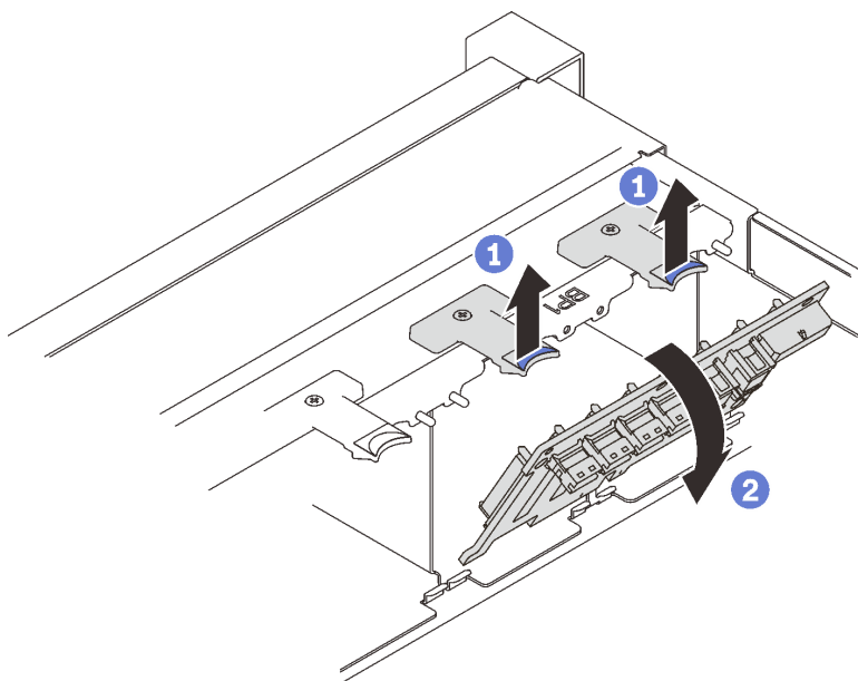
圖例 30. 卸下硬碟背板
