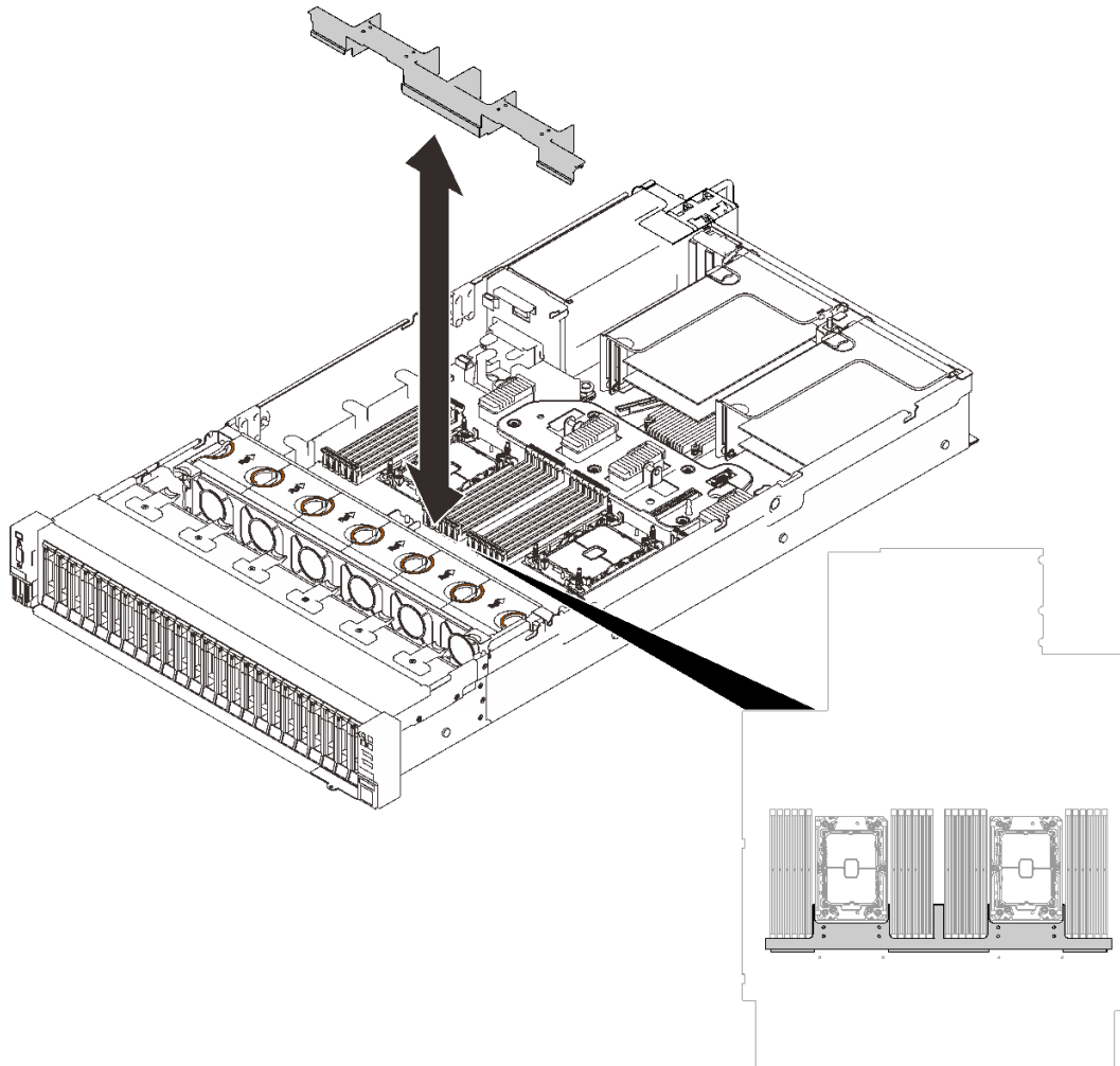
圖例 114. 安裝擴充匣空氣擋板
