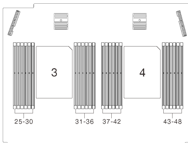
圖例 67. 擴充匣上的記憶體模組插槽 25-48
