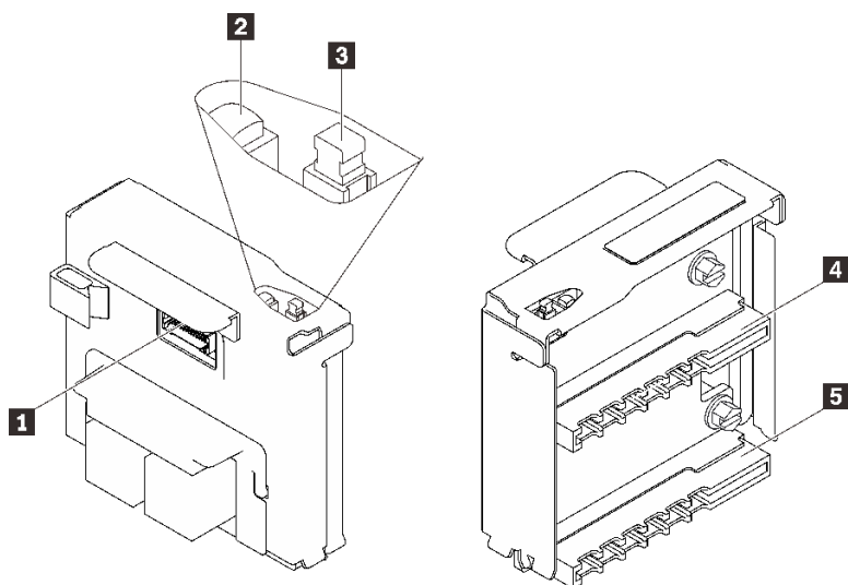
圖例 11. 電源背板元件
