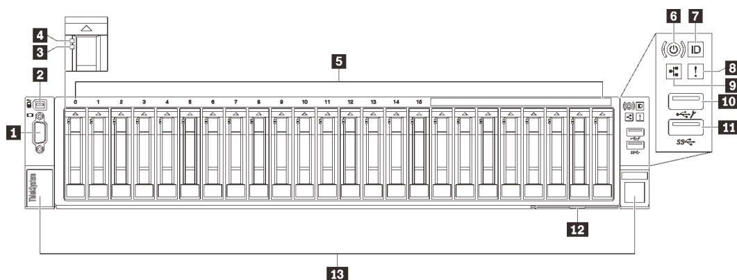
圖例 5. 正面圖
