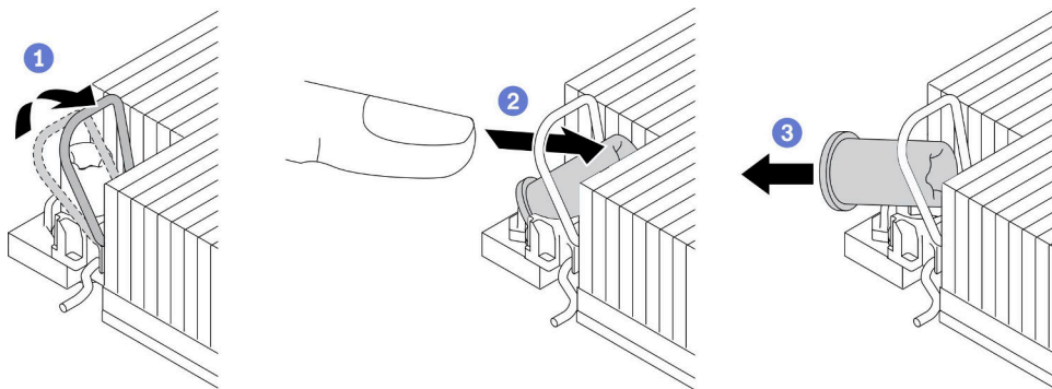
圖例 62. 從散熱槽卸下 Torx T30 螺帽
