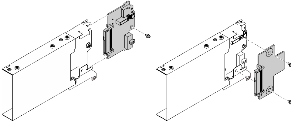
圖例 37. 拆卸 7 公釐框架
