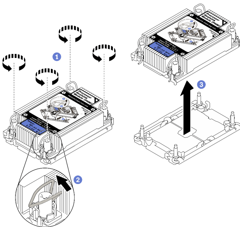
圖例 99. 卸下 PHM
