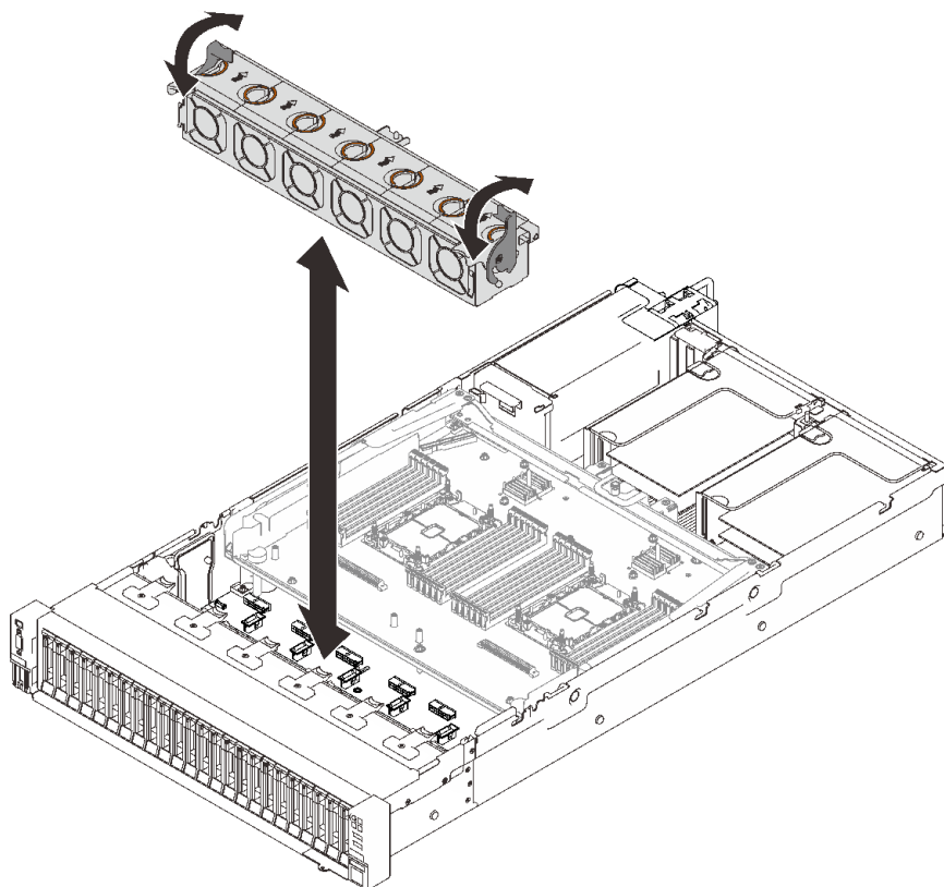
圖例 50. 安裝風扇機盒組件
