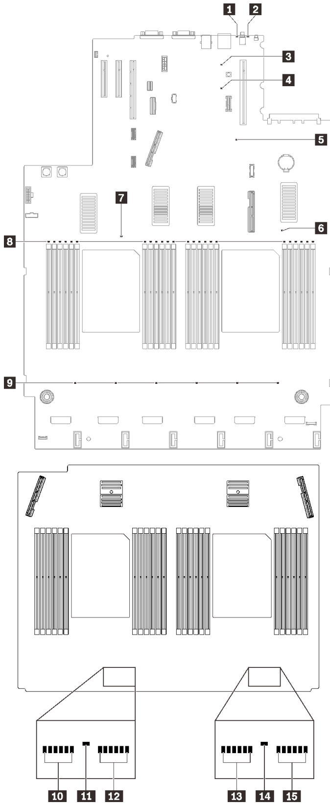
圖例 137. 主機板和擴充主機板 LED
