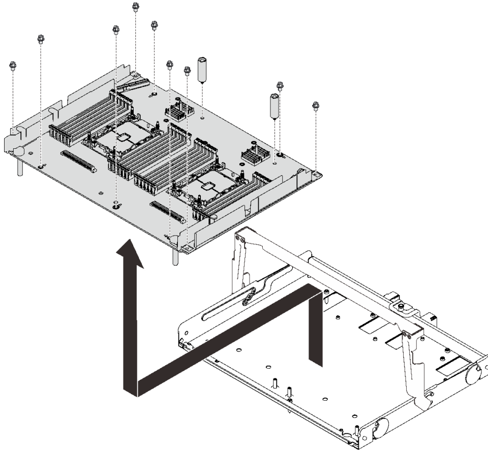
圖例 113. 拆卸擴充匣
