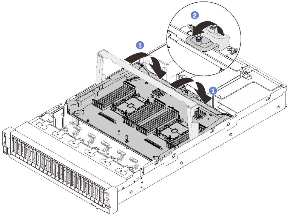
圖例 117. 固定處理器和記憶體擴充匣
