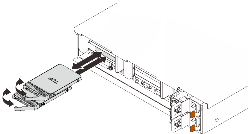
圖例 41. 安裝 7 公釐硬碟
