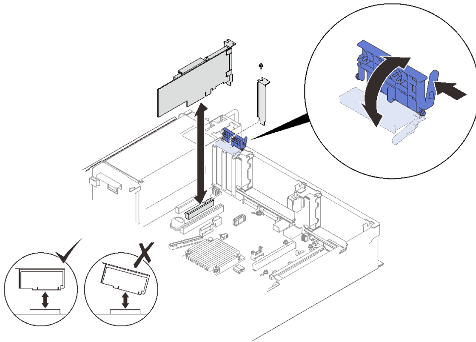
圖例 77. 從主機板卸下配接卡
