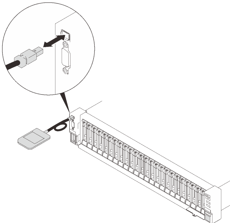
圖例 47. 連接外部 LCD 診斷手持裝置纜線
