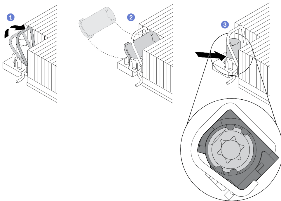
圖例 63. 將 Torx T30 螺帽安裝到散熱槽
