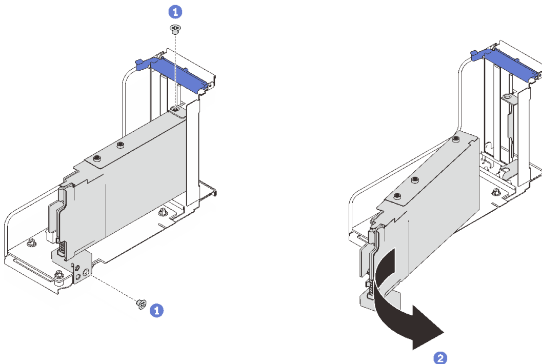
圖例 36. 從擴充卡卸下 7 公釐框架
