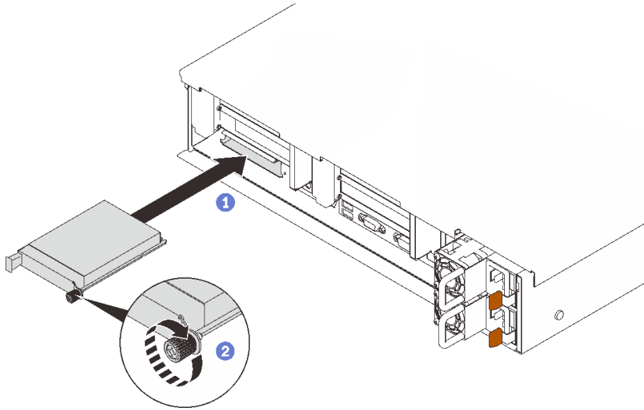
圖例 73. 安裝 OCP 乙太網路配接卡
