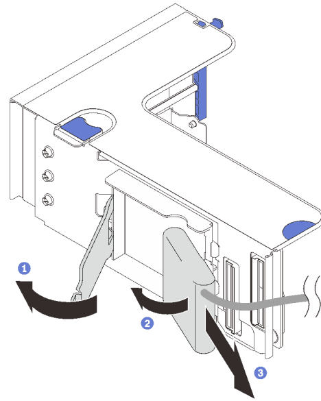
圖例 54. 從水平固定器卸下快閃記憶體電源模組
