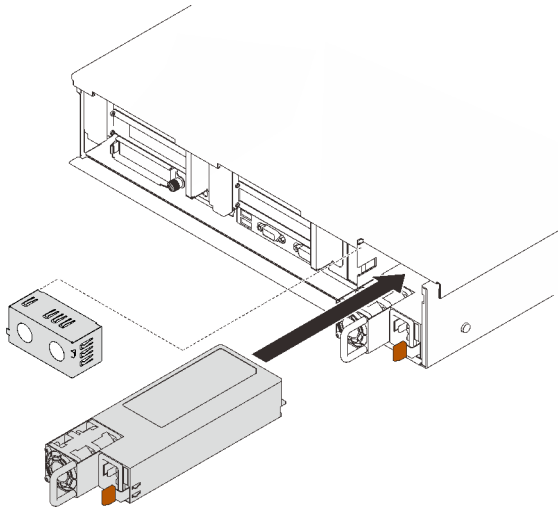
圖例 92. 安裝電源供應器
