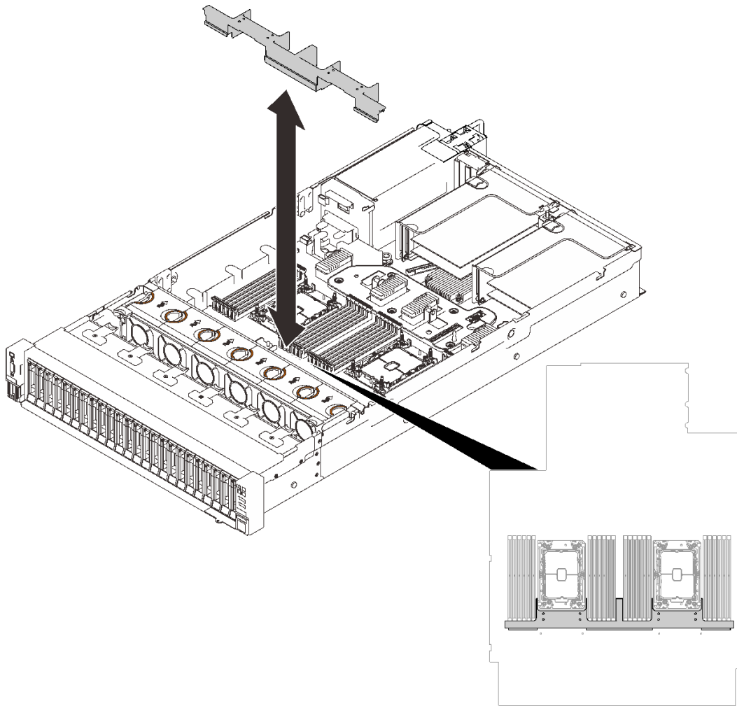
圖例 24. 安裝擴充匣空氣擋板
