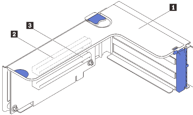
圖例 14. x16/x16 ( x8 通道 ) PCIe 擴充卡接頭
