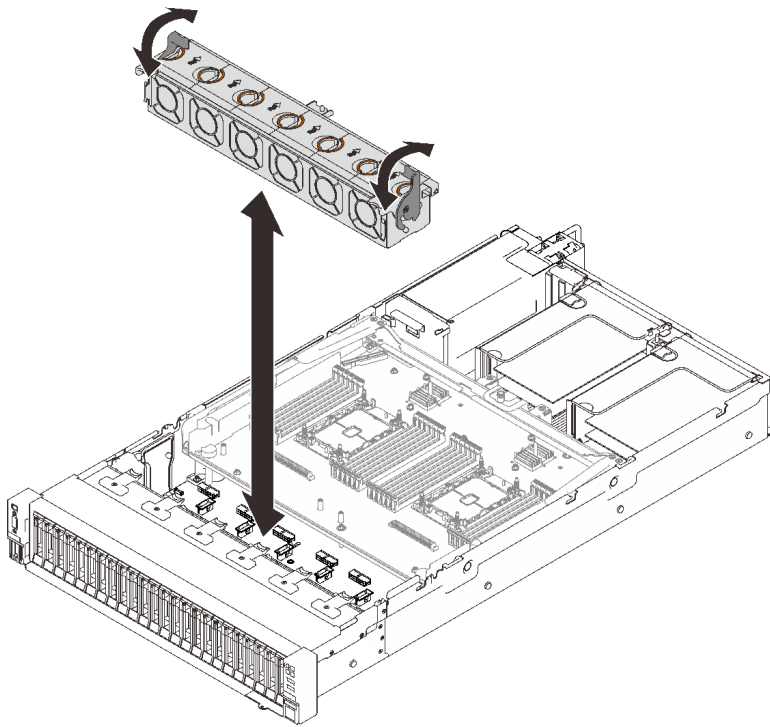
圖例 49. 卸下風扇機盒組件
