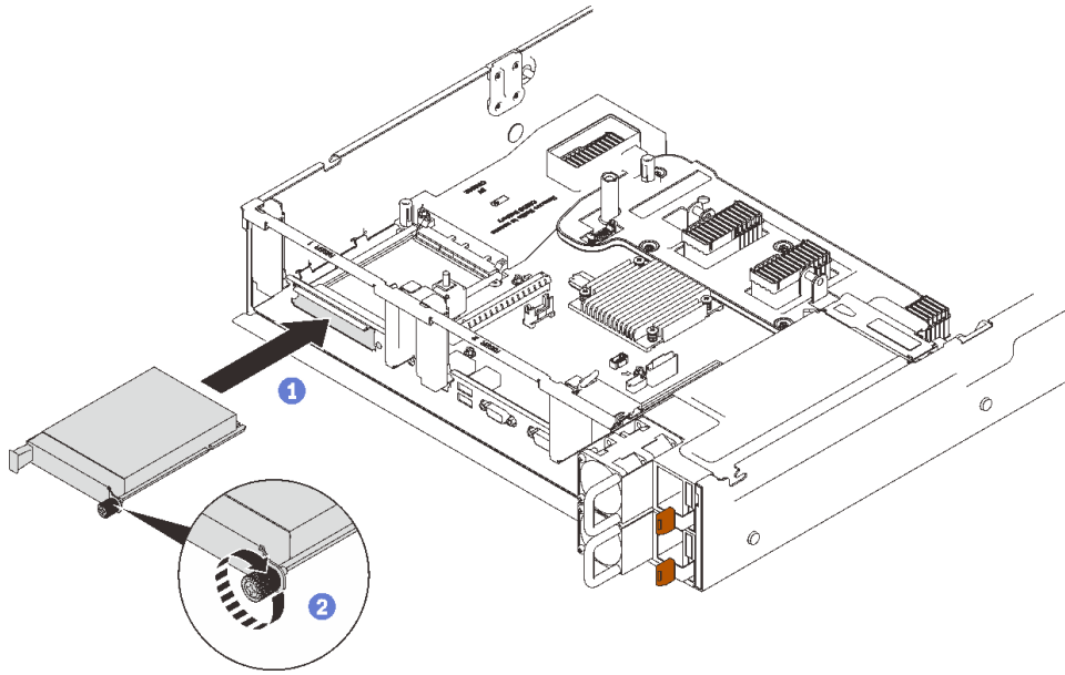
圖例 67. 安裝 OCP 乙太網路配接卡
