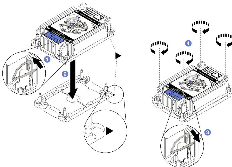
圖例 79. 安裝 PHM
