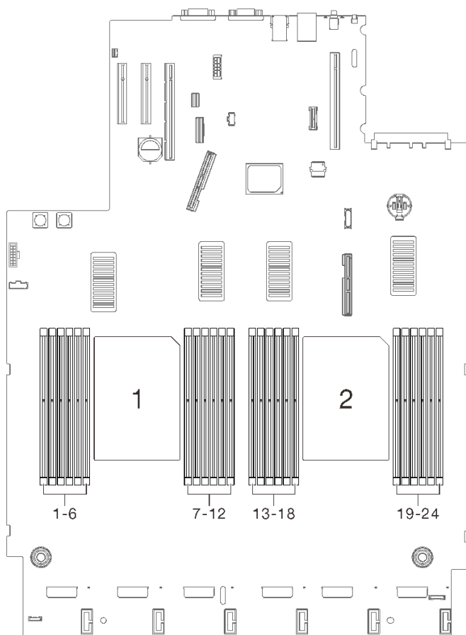
圖例 76. 主機板上的處理器 1 和 2 位置
