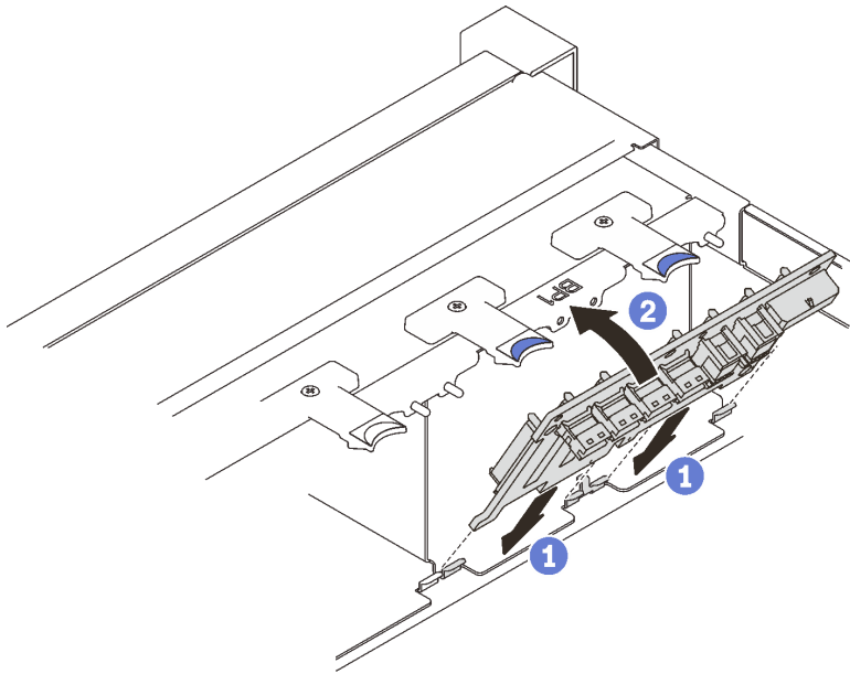
圖例 55. 安裝硬碟背板
