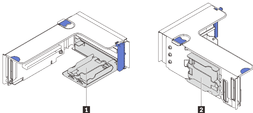
圖例 61. 快閃記憶體電源模組匣
