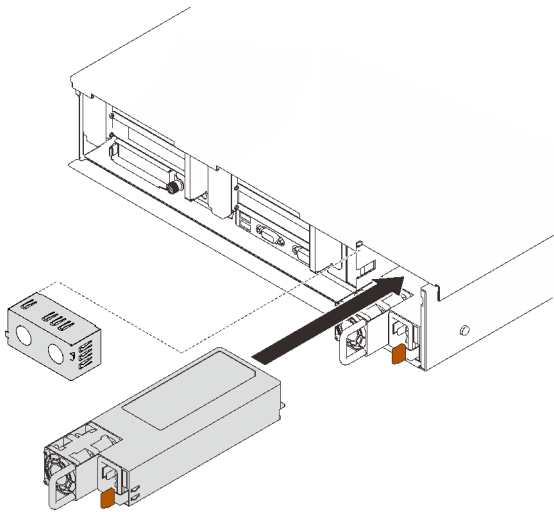
圖例 50. 安裝電源供應器
