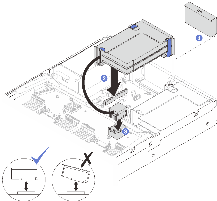
圖例 70. 將 PCIe 擴充卡組件安裝到區域 2
