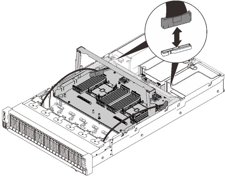
圖例 73. 拔掉 PCIe 纜線
