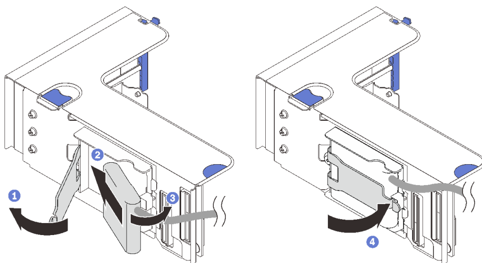
圖例 63. 安裝快閃記憶體電源模組
