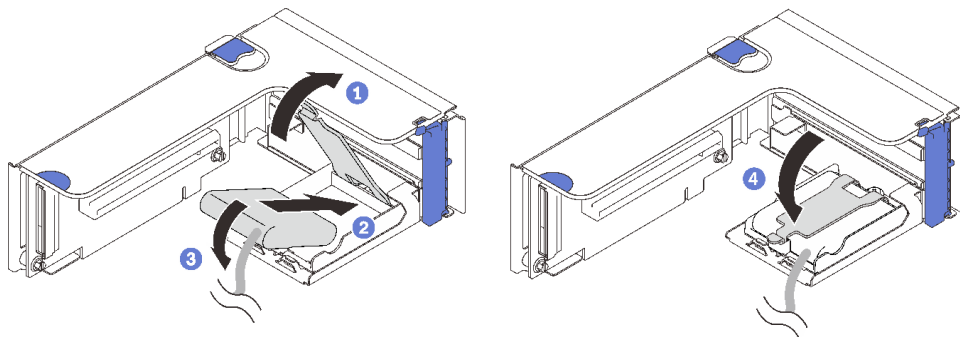
圖例 65. 安裝快閃記憶體電源模組
