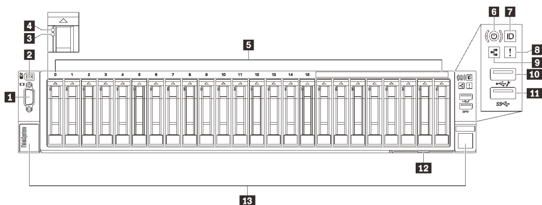
圖例 5. 正面圖
