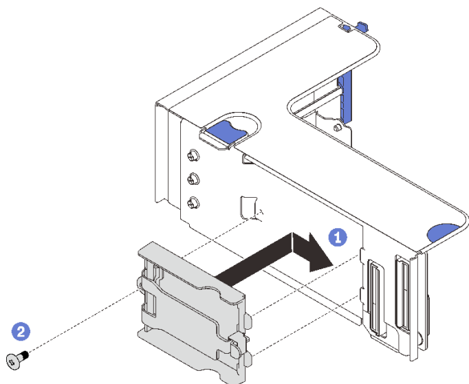
圖例 62. 安裝垂直匣
