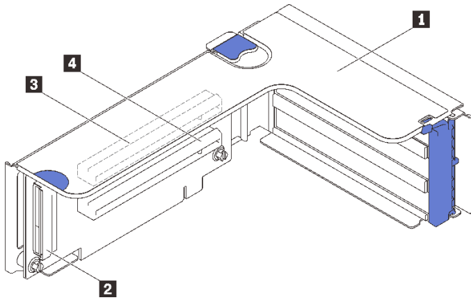
圖例 42. x16/x16 PCIe 擴充卡接頭
