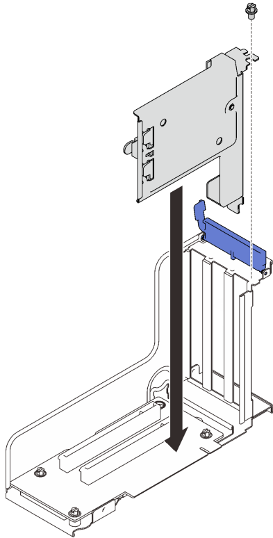
圖例 64. 將快閃記憶體電源模組托架安裝到擴充卡中
