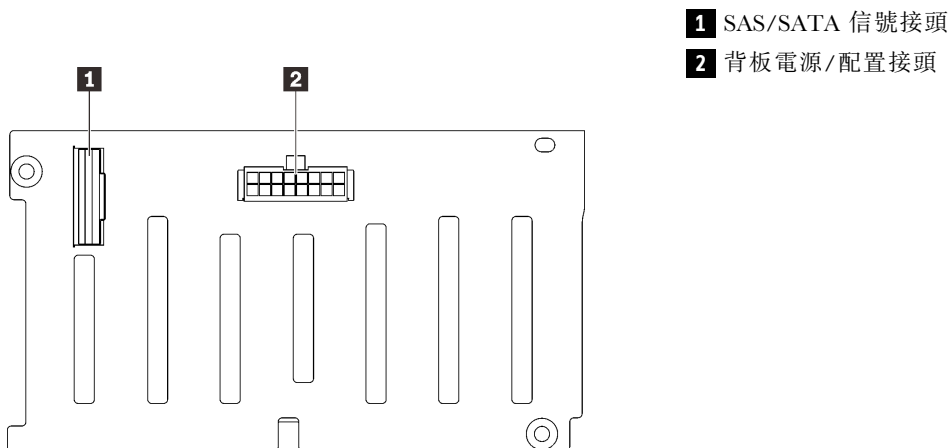
圖例 28. SAS/SATA 硬碟背板接頭
