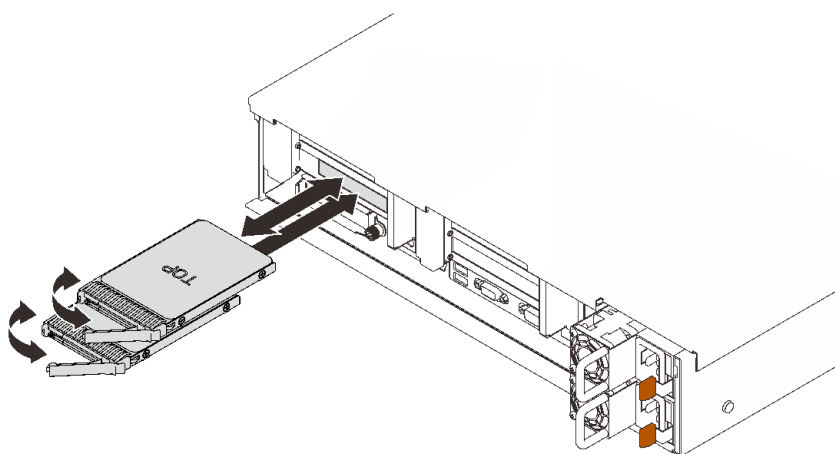
圖例 46. 安裝 7 公釐硬碟
