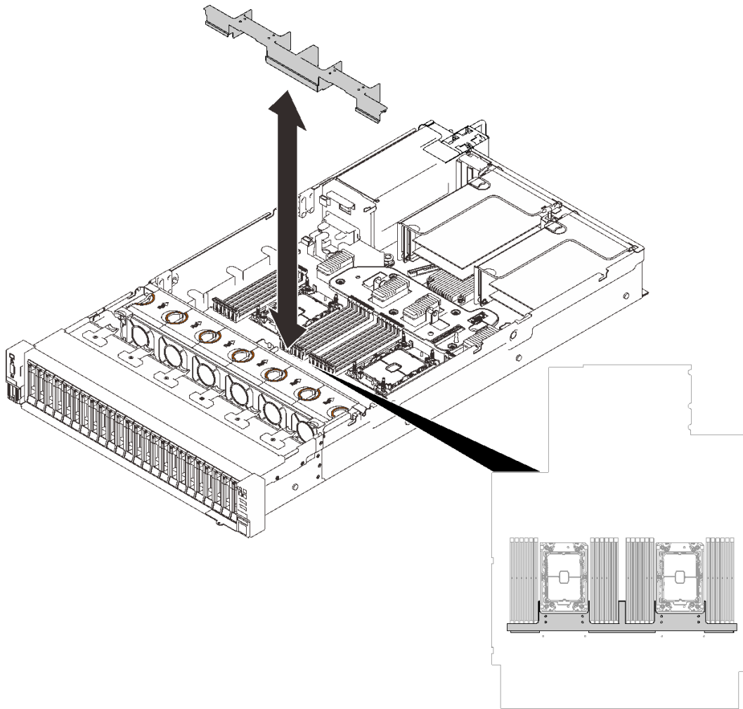
圖例 83. 安裝擴充匣空氣擋板
