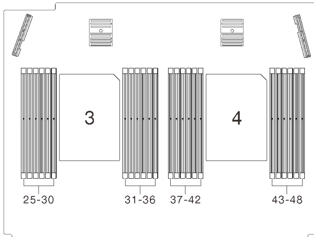
圖例 77. 處理器和記憶體擴充匣上的處理器 3 和 4 位置
