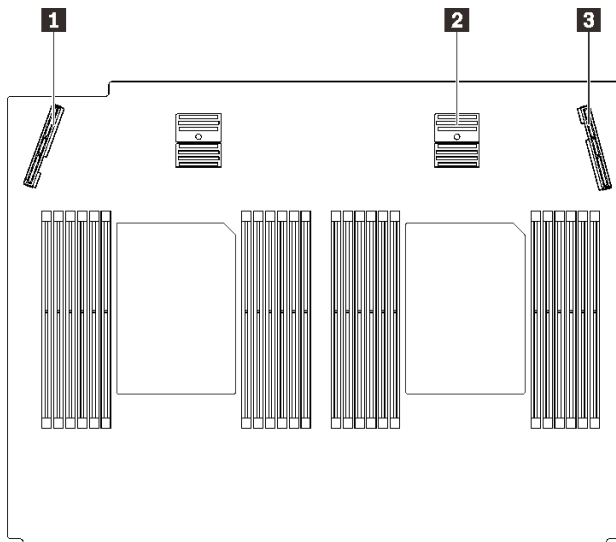
圖例 44. 處理器和記憶體擴充匣接頭
