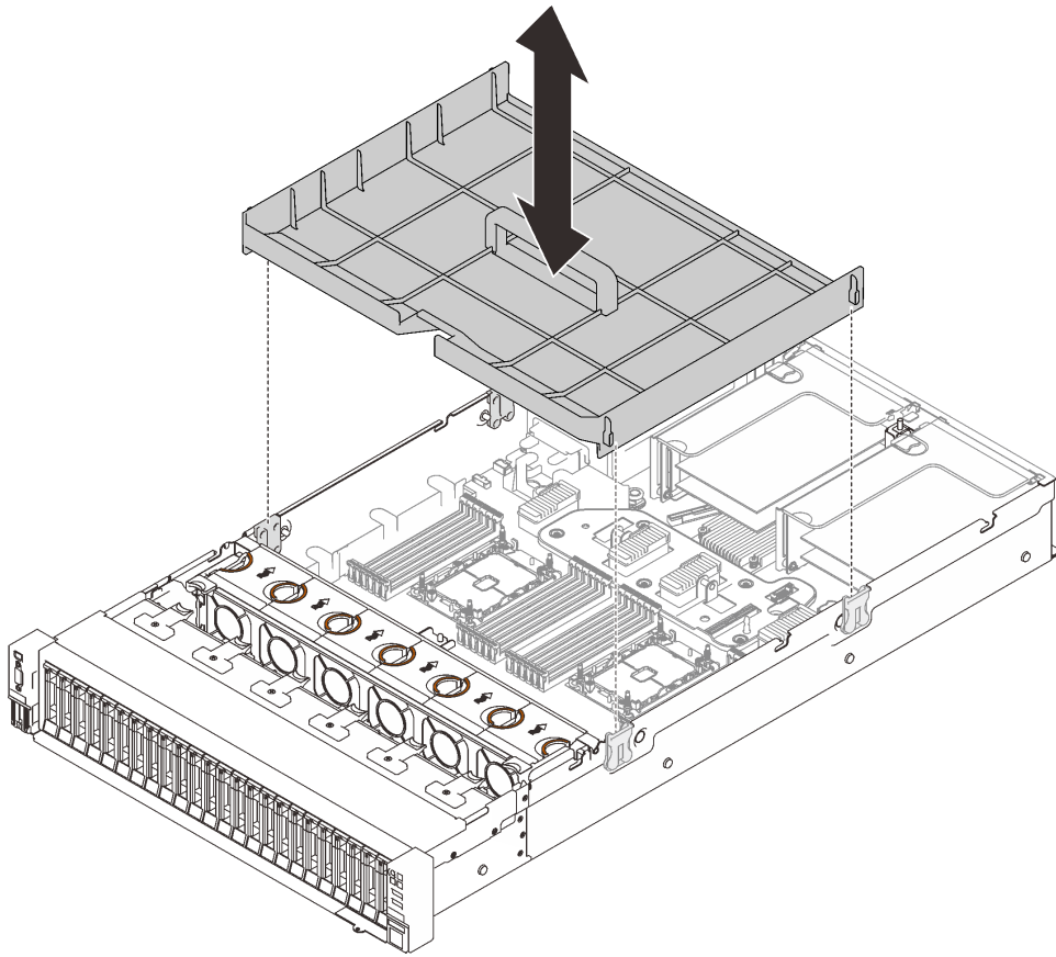
圖例 71. 卸下主機板空氣擋板
