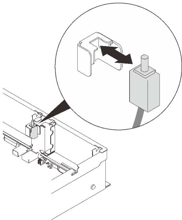
圖例 56. 安裝入侵開關
