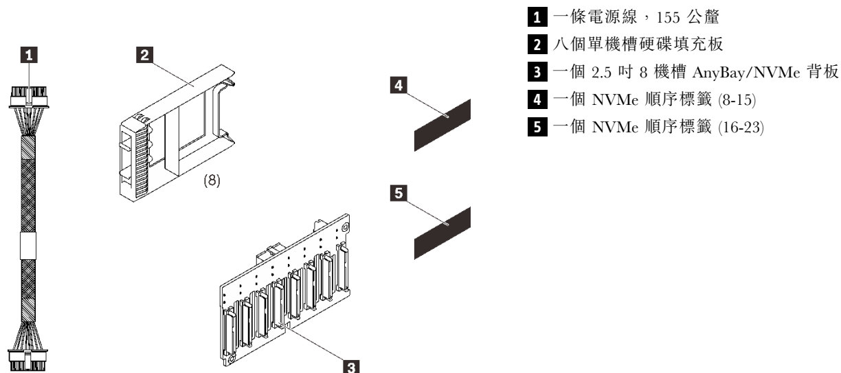
圖例 29. 2.5 吋 8 機槽 SAS/SATA 背板套件
