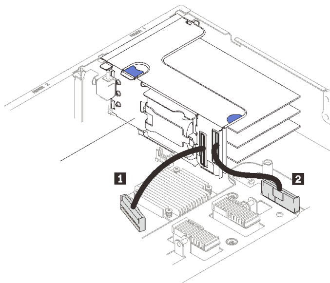
圖例 69. 將 PCIe 纜線從 x16/x16/x16 擴充卡連接到主機板
