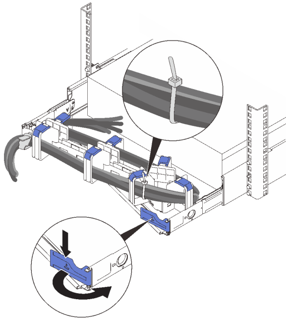
圖例 49. 調整 CMA
