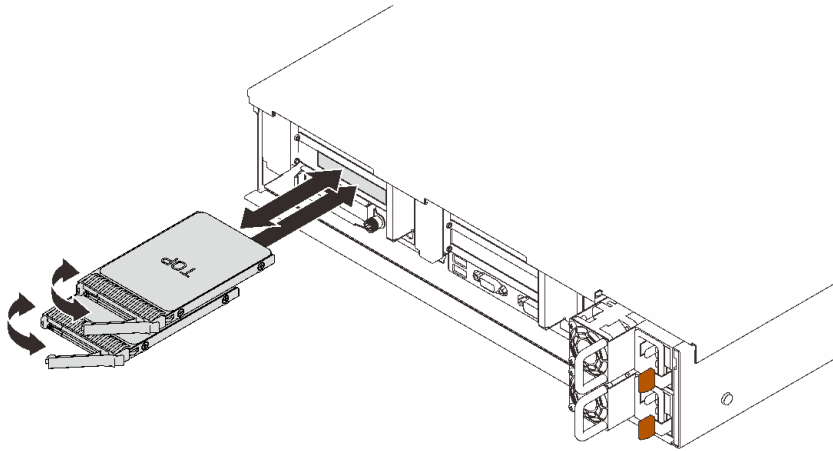
圖例 53. 卸下 7 公釐硬碟
