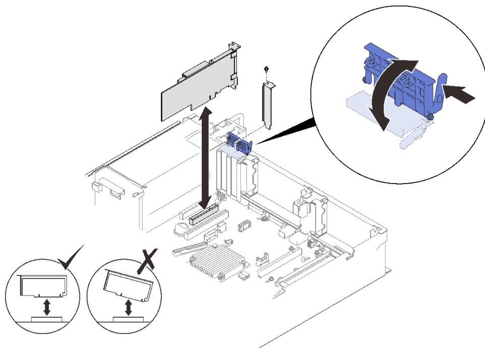
圖例 59. 將配接卡安裝到主機板
