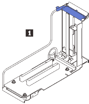
圖例 35. x16/x16 ( x8 通道 ) FH/HL PCIe 擴充卡套件
