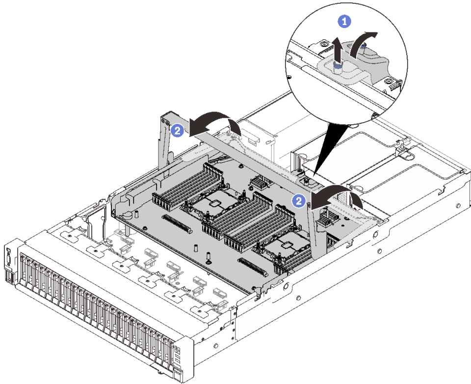
圖例 72. 鬆開處理器和記憶體擴充匣
