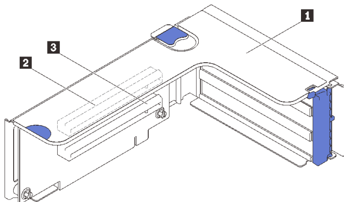
圖例 14. x16/x16 ( x8 通道 ) PCIe 擴充卡接頭
