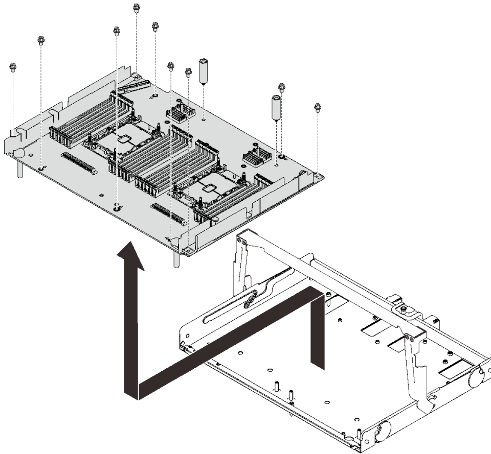
圖例 75. 拆卸擴充匣
