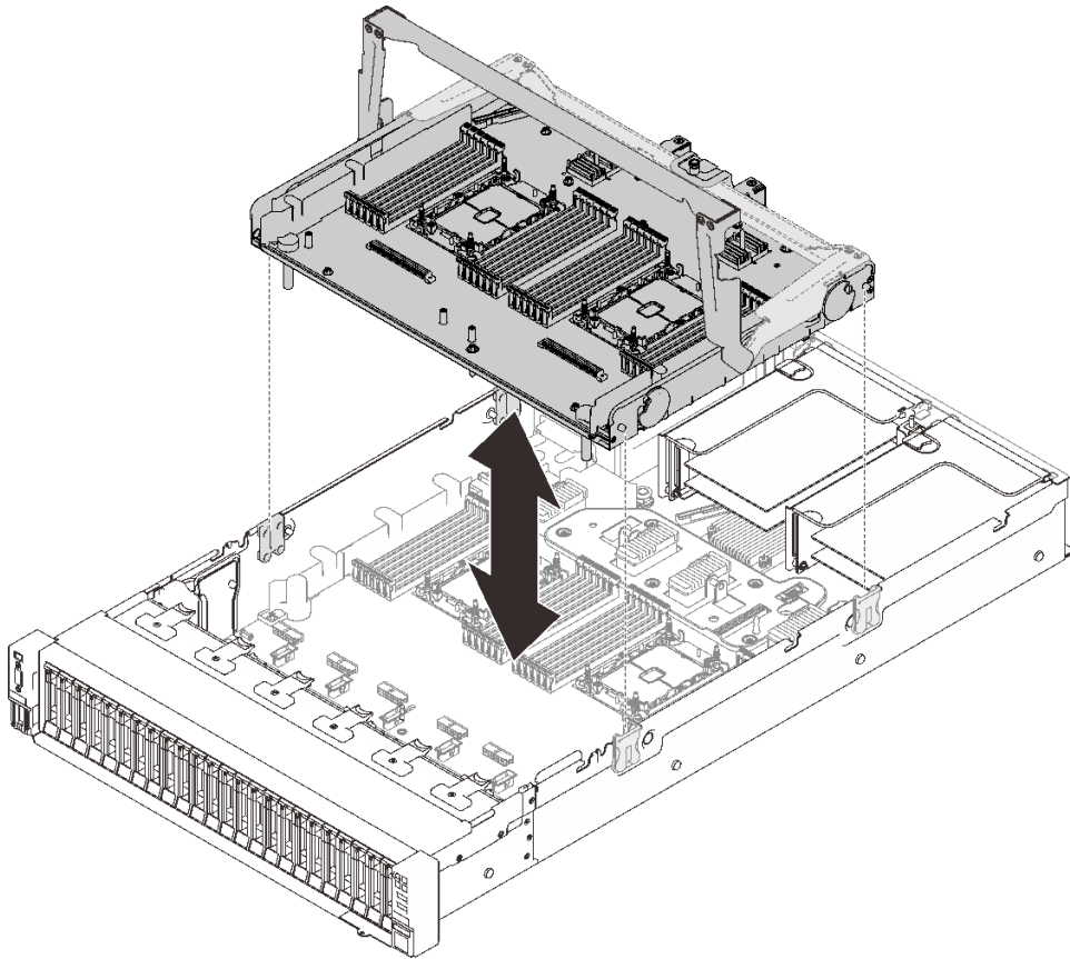
圖例 74. 卸下處理器和記憶體擴充匣
