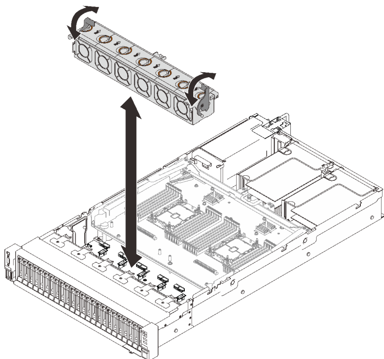
圖例 54. 卸下風扇機盒組件
