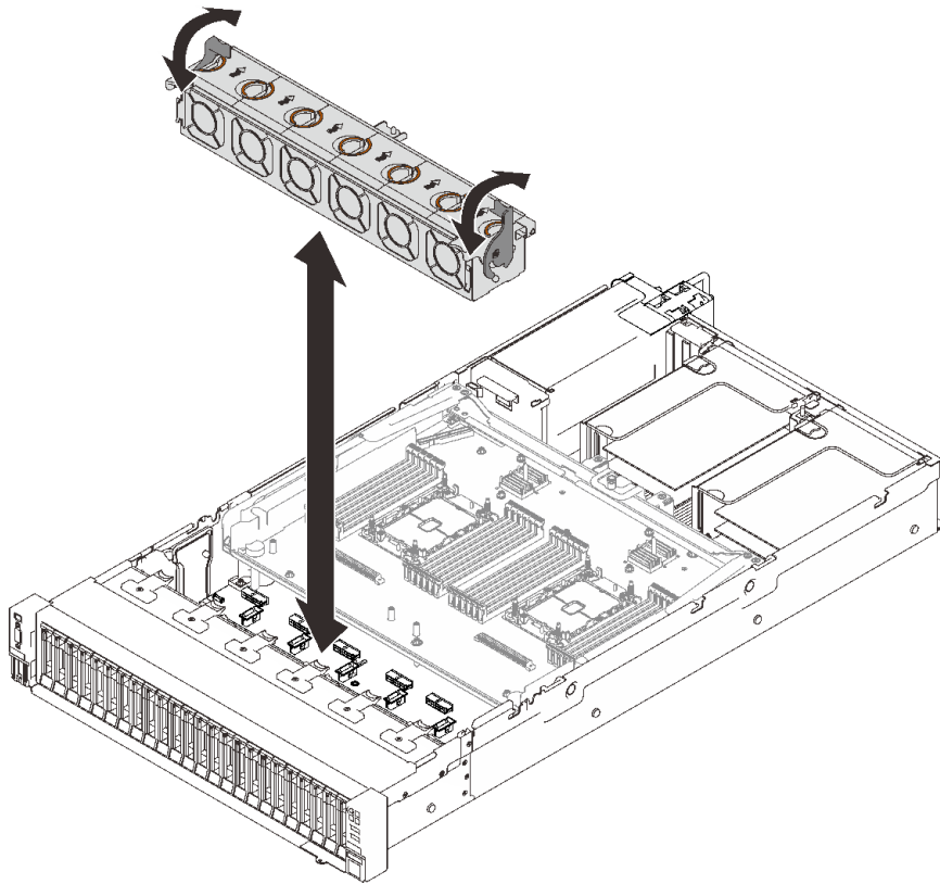
圖例 87. 安裝風扇機盒組件
