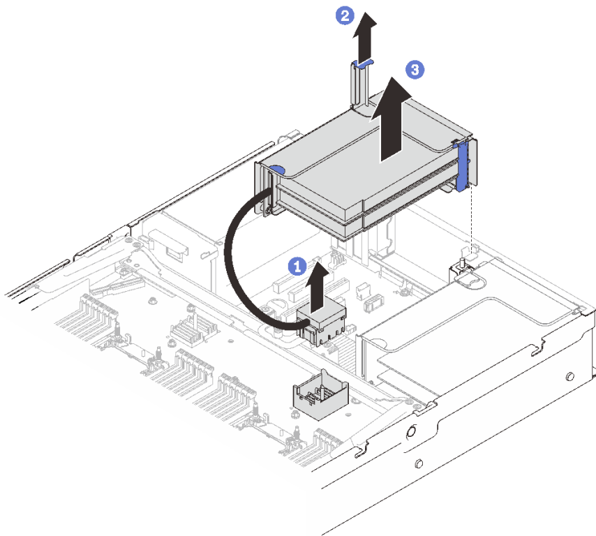
圖例 58. 從區域 2 卸下 PCIe 擴充卡組件
