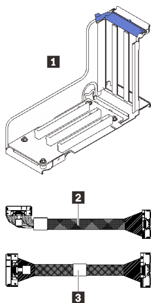
圖例 39. x16/x16/x16 PCIe 擴充卡
