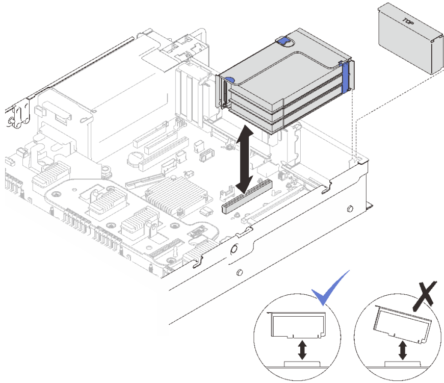
圖例 57. 從區域 1 卸下 PCIe 擴充卡組件
