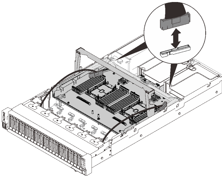
圖例 23. 將纜線連接到擴充匣
