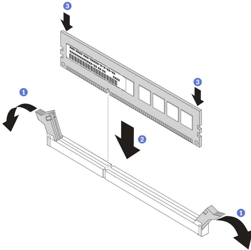
圖例 80. 安裝記憶體模組
