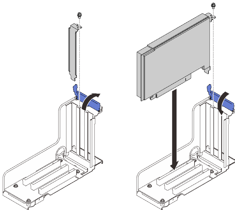
圖例 60. 將配接卡安裝到 PCIe 擴充卡組件中
