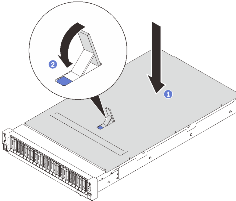
圖例 88. 安裝上蓋
