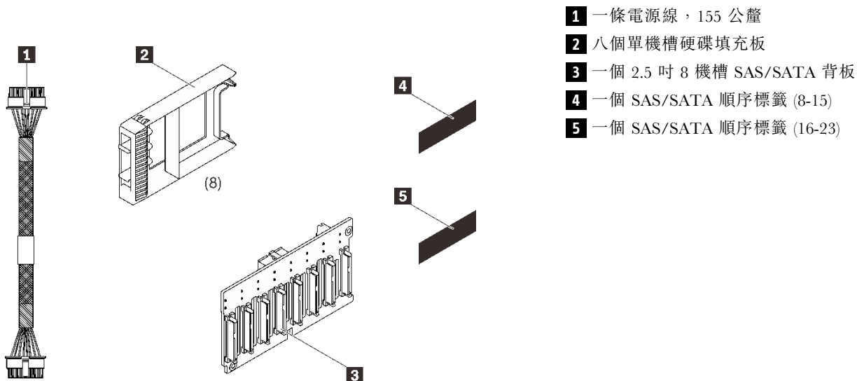
圖例 27. 2.5 吋 8 機槽 SAS/SATA 背板套件
