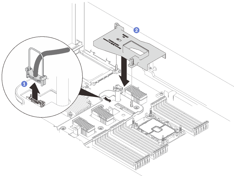
圖例 66. 安裝 OCP 配接卡空氣擋板
