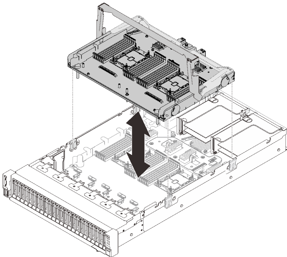
圖例 84. 安裝處理器和記憶體擴充匣
