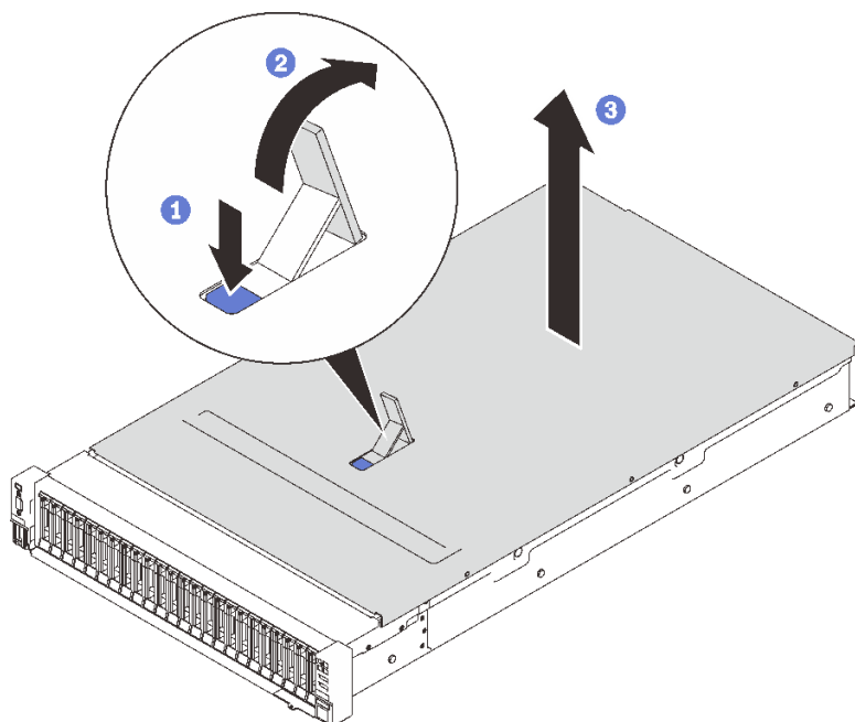
圖例 52. 卸下上蓋
