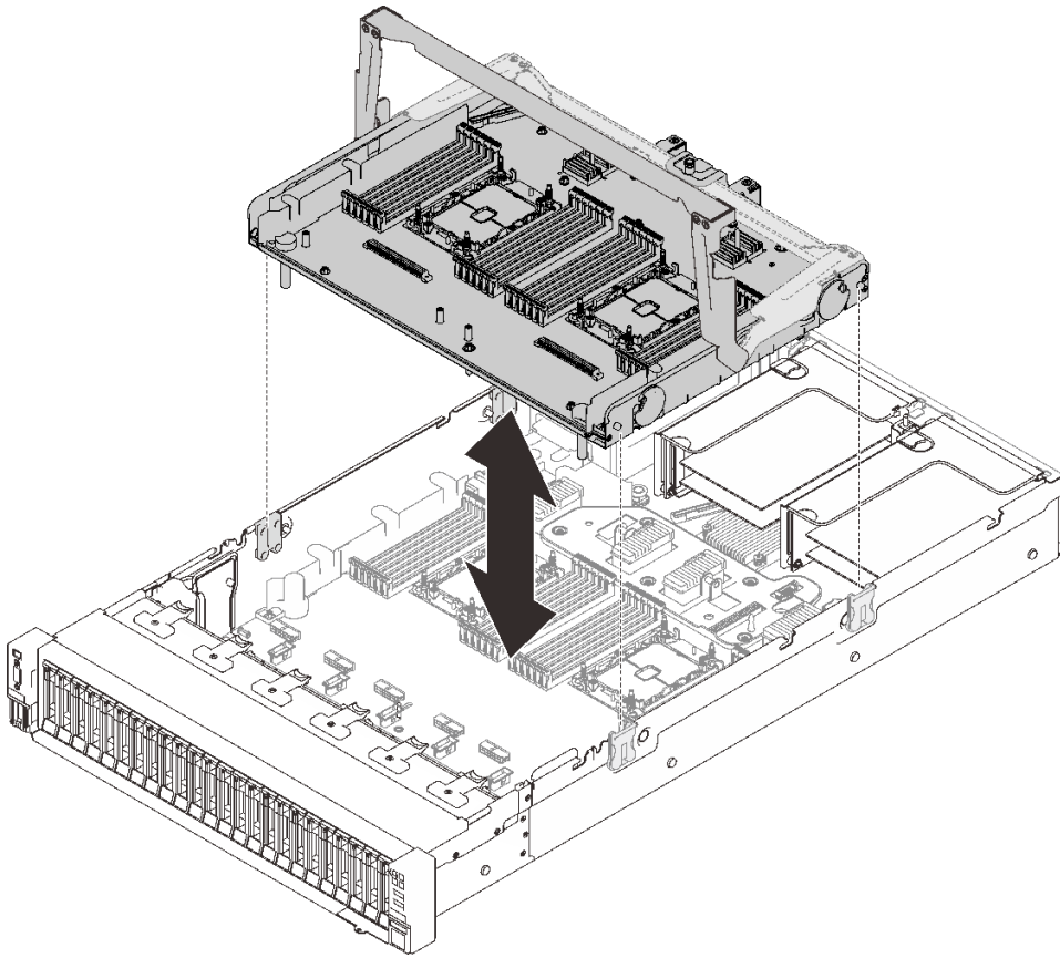
圖例 22. 安裝處理器和記憶體擴充匣
