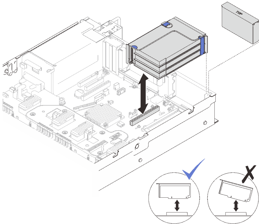
圖例 68. 將 PCIe 擴充卡組件安裝到區域 1
