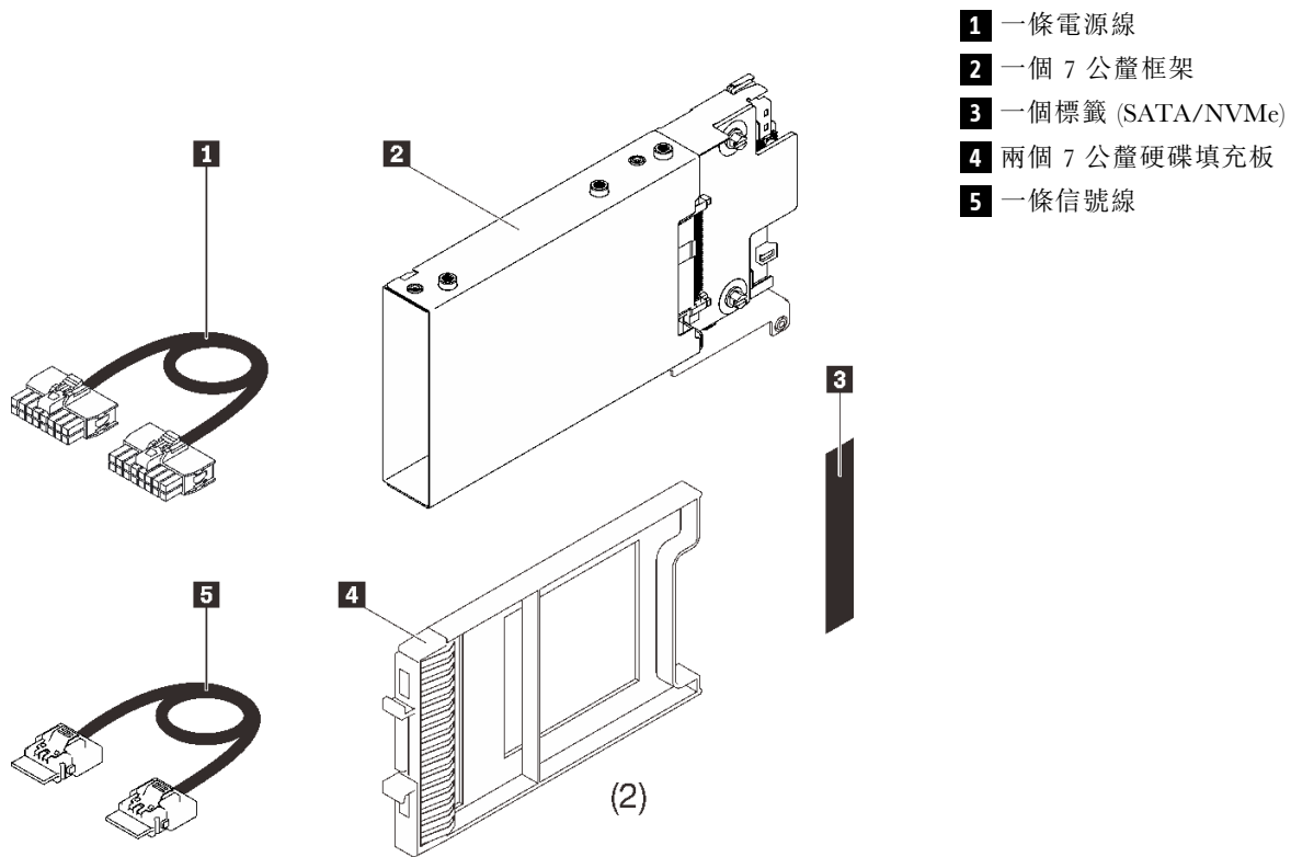
圖例 34. 7 公釐框架套件
