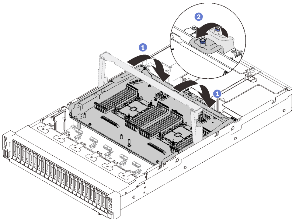
圖例 86. 固定處理器和記憶體擴充匣
