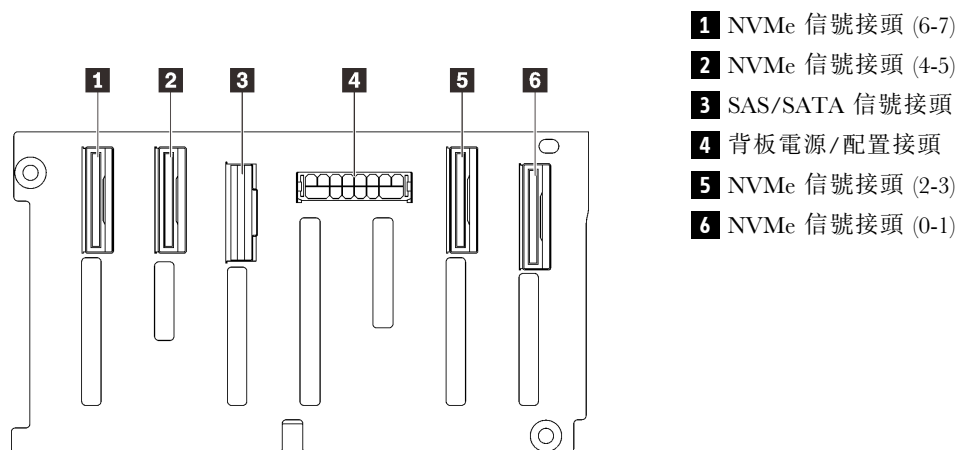
圖例 30. AnyBay/NVMe 硬碟背板接頭
