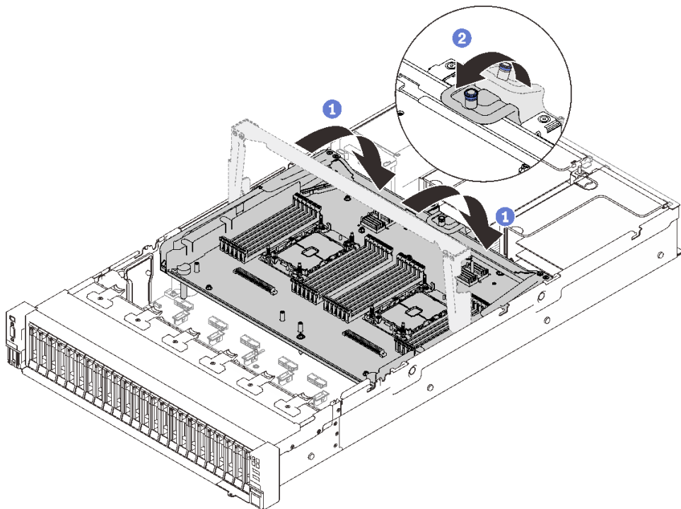
圖例 24. 固定處理器和記憶體擴充匣
