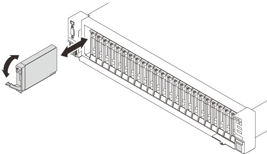
圖例 48. 安裝 2.5 吋硬碟
