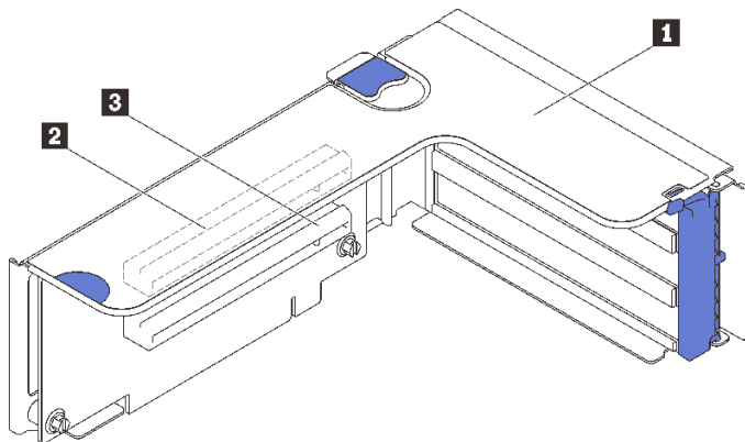
圖例 36. x16/x16 ( x8 通道 ) PCIe 擴充卡接頭
