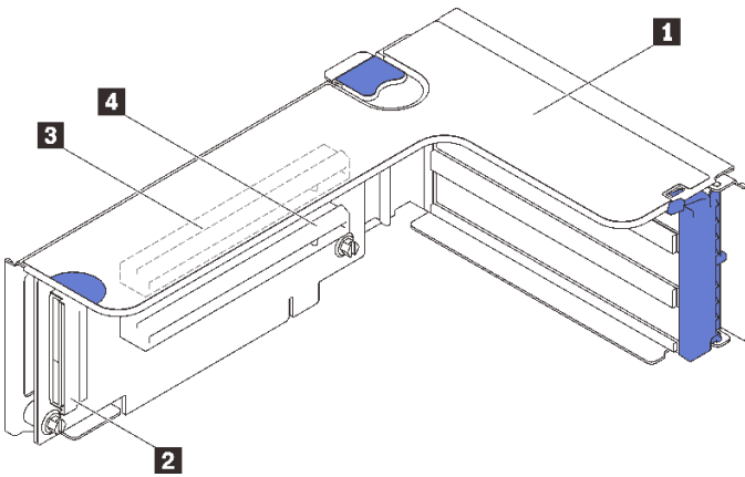
圖例 38. x16/x16 PCIe 擴充卡接頭
