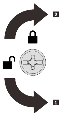
圖例 89. 上蓋鎖定/解鎖方向
