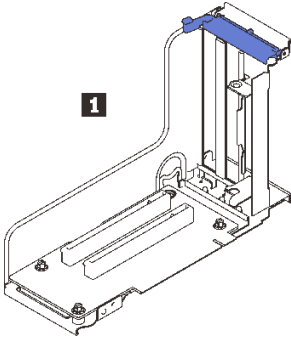
圖例 37. x16/x16 ( x8 通道 ) FH/HL PCIe 擴充卡
