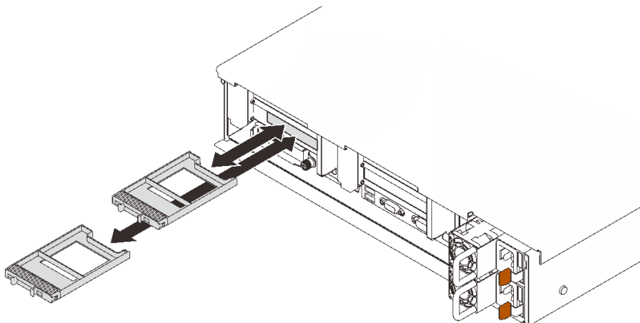
圖例 45. 卸下 7 公釐硬碟填充板
