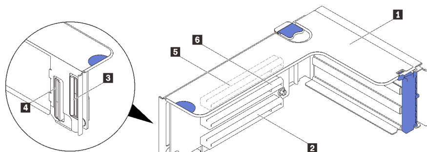
圖例 40. x16/x16/x16 PCIe 擴充卡接頭
