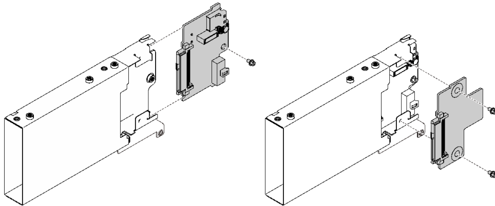
圖例 81. 安裝 7 公釐硬碟背板
