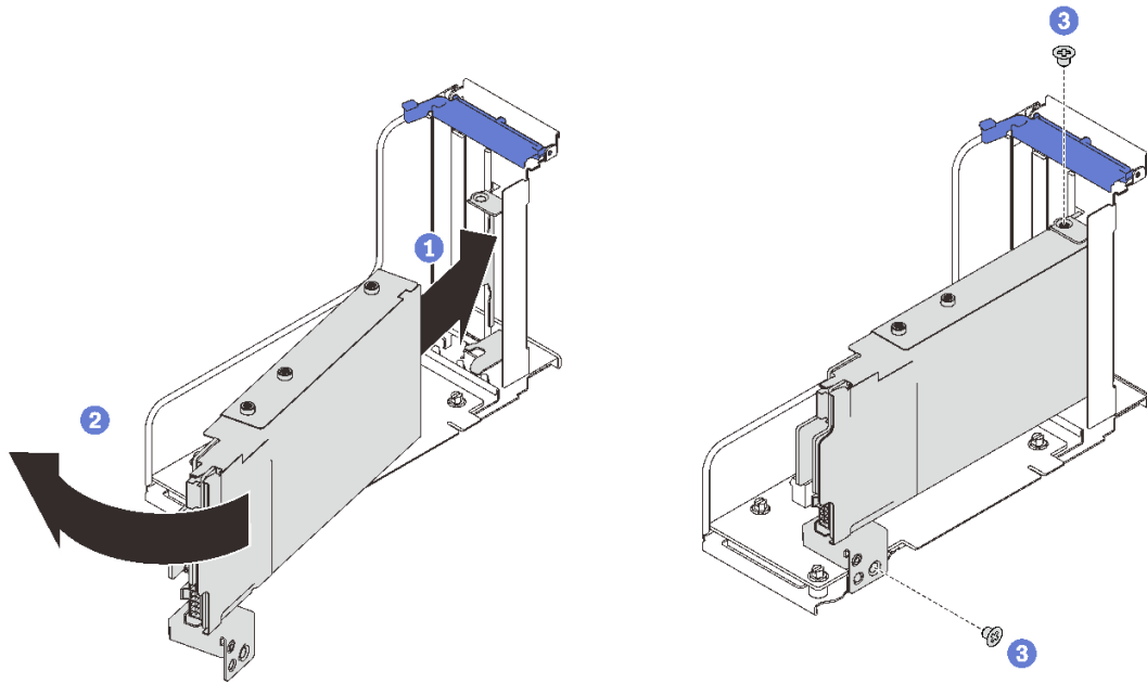
圖例 82. 將 7 公釐框架安裝到擴充卡
