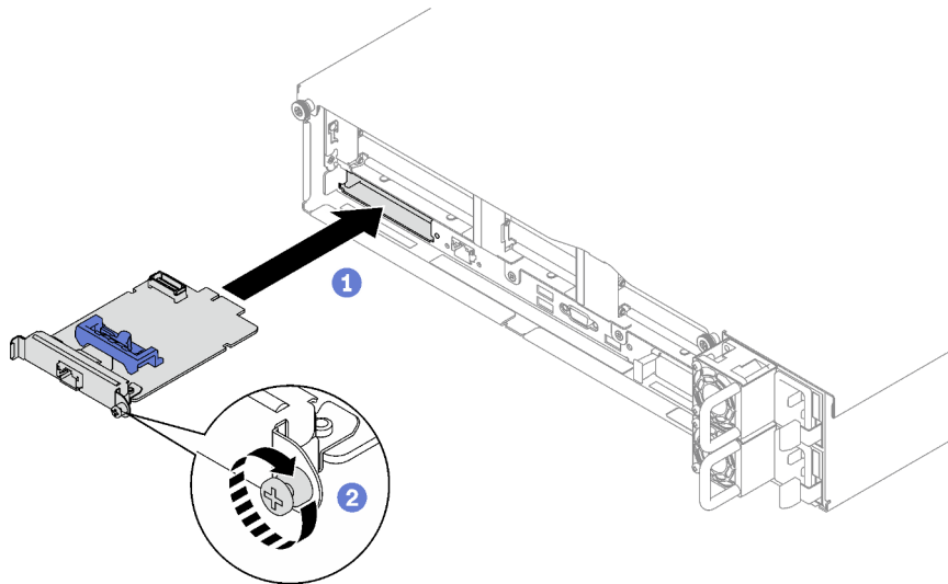
Figura 64. Instalación del Adaptador NIC de gestión
