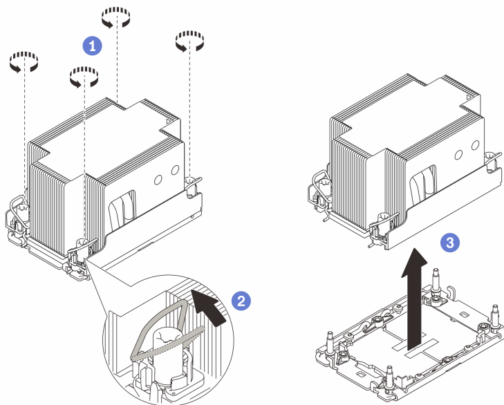
Figura 110. Extracción del PHM estándar 2U
