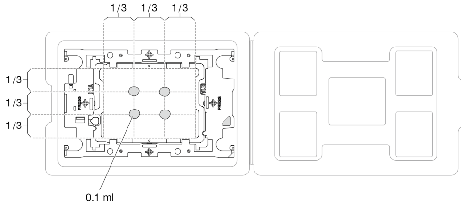
Figura 116. Aplicación de grasa térmica con el procesador en la bandeja de envío
