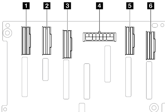
Figura 143. 8 conectores de placa posterior SAS/SATA/NVMe de 2,5 pulgadas
