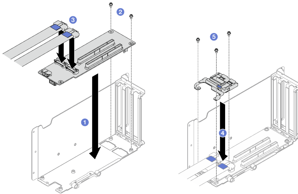
Figura 92. Instalación de la tarjeta de expansión PCIe
