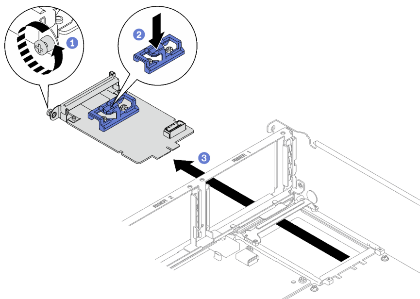
Figura 63. Extracción del Adaptador NIC de gestión
