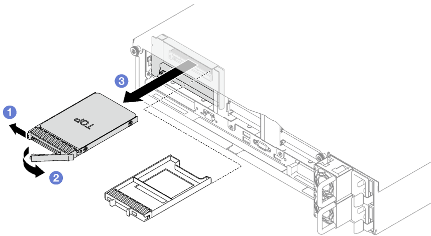
Figura 8. Extracción de una unidad de 7 mm
