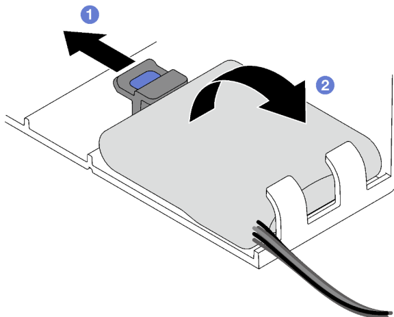
Figura 43. Extracción del módulo de alimentación flash
