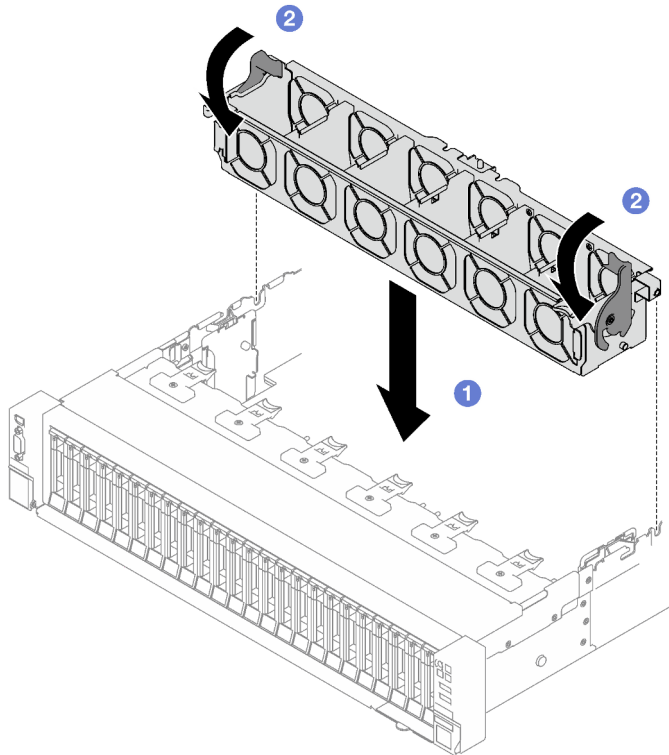
Figura 40. Instalación de la caja del ventilador
