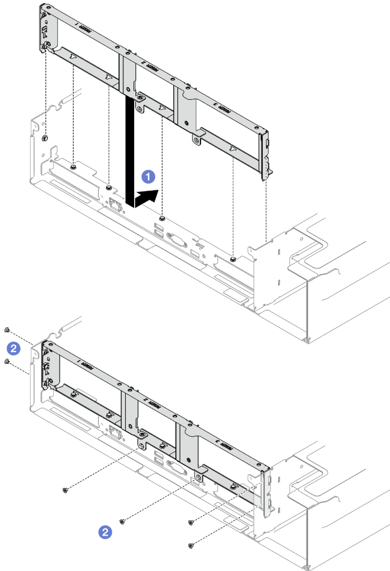
Figura 121. Instalación del muro posterior
