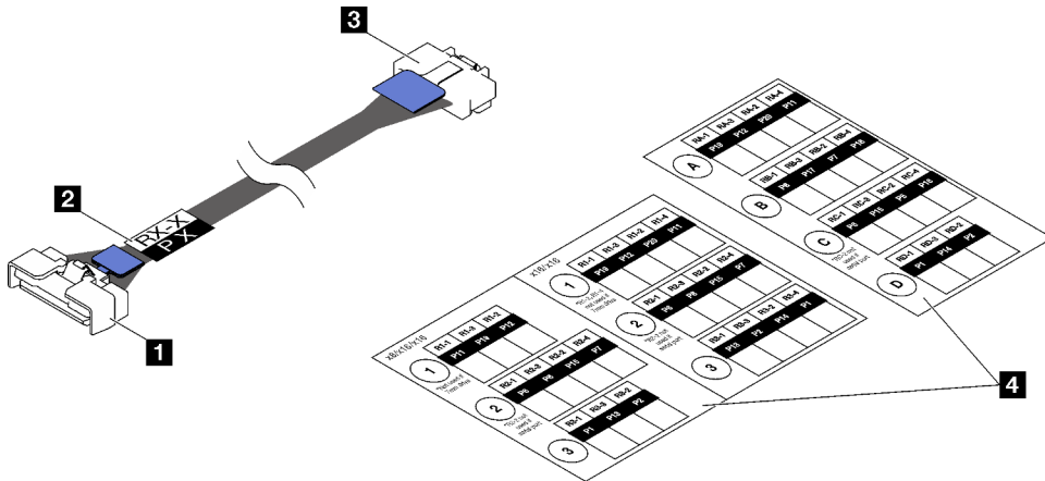
Figura 89. Cable de expansión PCIe
