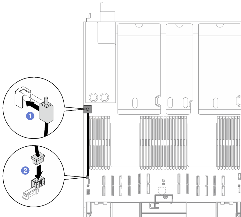
Figura 52. Instalación del conmutador de intrusión
