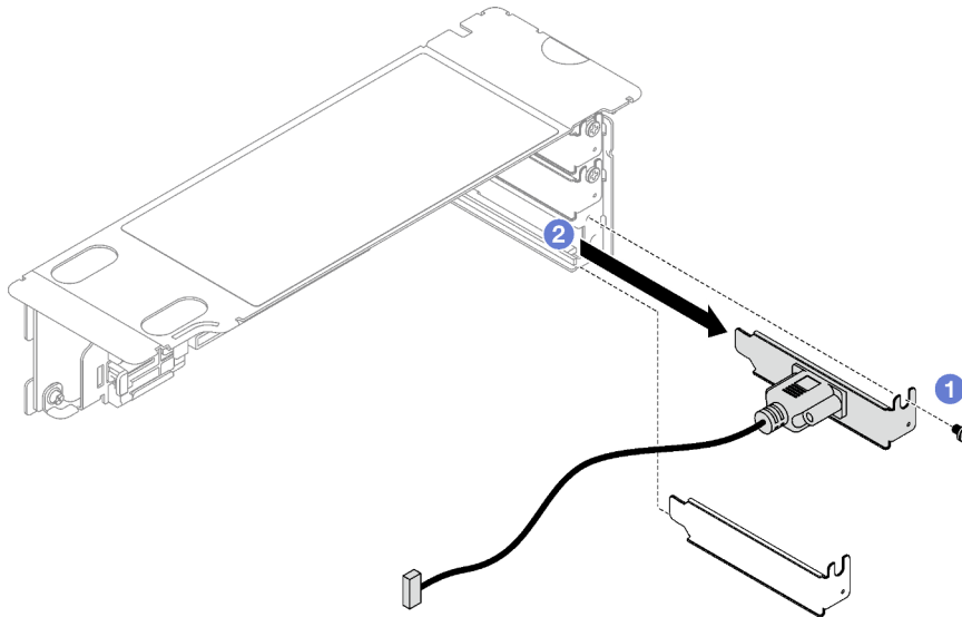
Figura 126. Extracción del módulo de puerto serie
