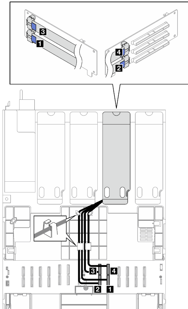
Figura 170. Disposición de cables para la expansión PCIe B
