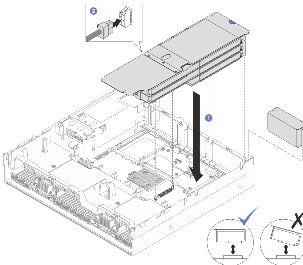
Figura 84. Instalación de expansión PCIe de FHFL
