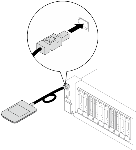
Figura 36. Conexión del cable del auricular de diagnóstico externo
