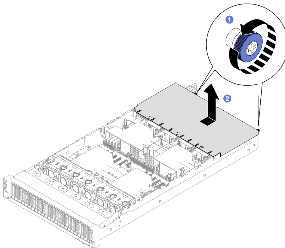
Figura 138. Extracción de la cubierta superior posterior
