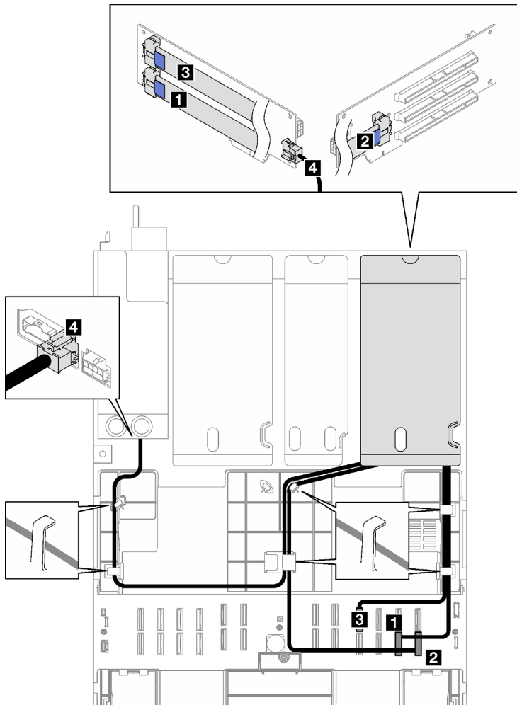
Figura 163. Disposición de cables para la expansión de tres ranuras PCIe de HL 1
