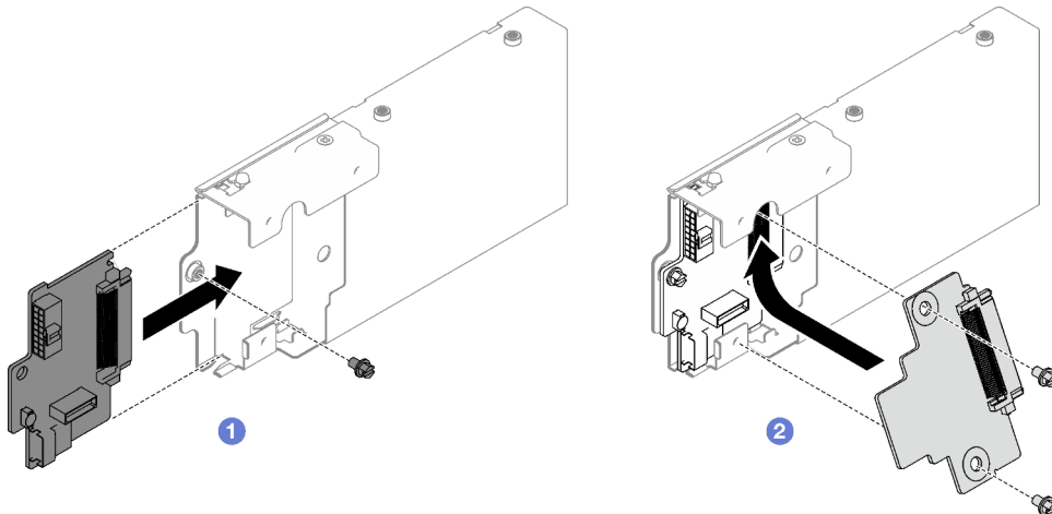
Figura 11. Instalación de una placa posterior de unidad de 7 mm
