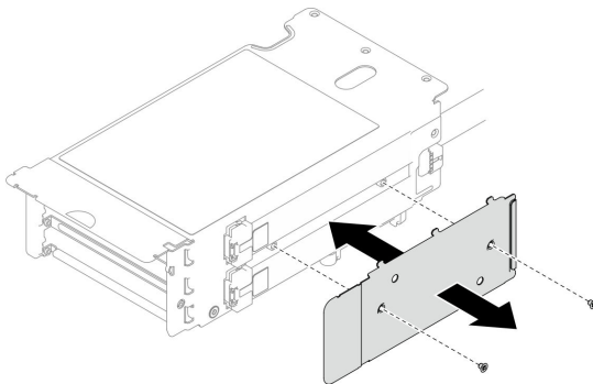
Figura 85. Extracción de la cubierta del cable
