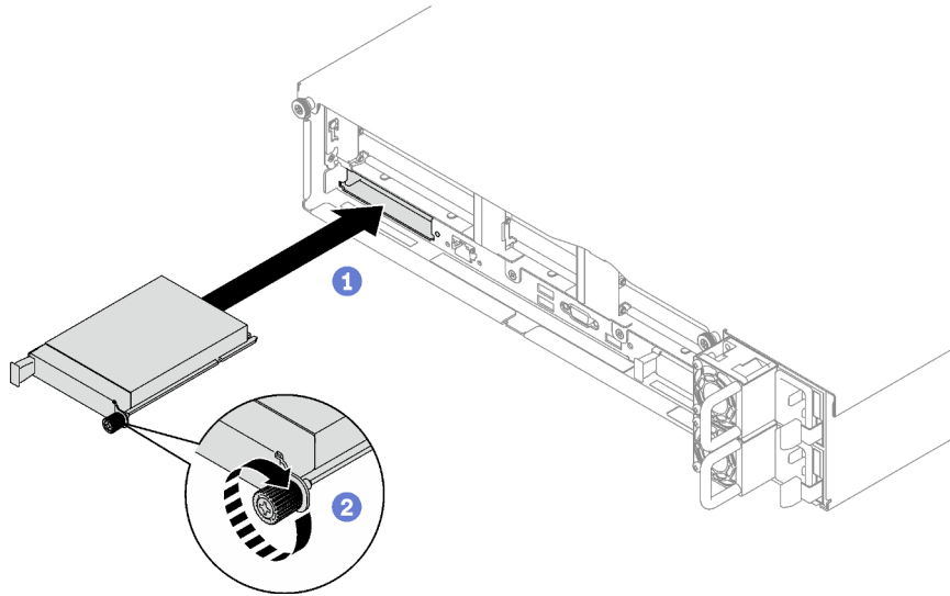
Figura 72. Instalación del módulo de OCP
