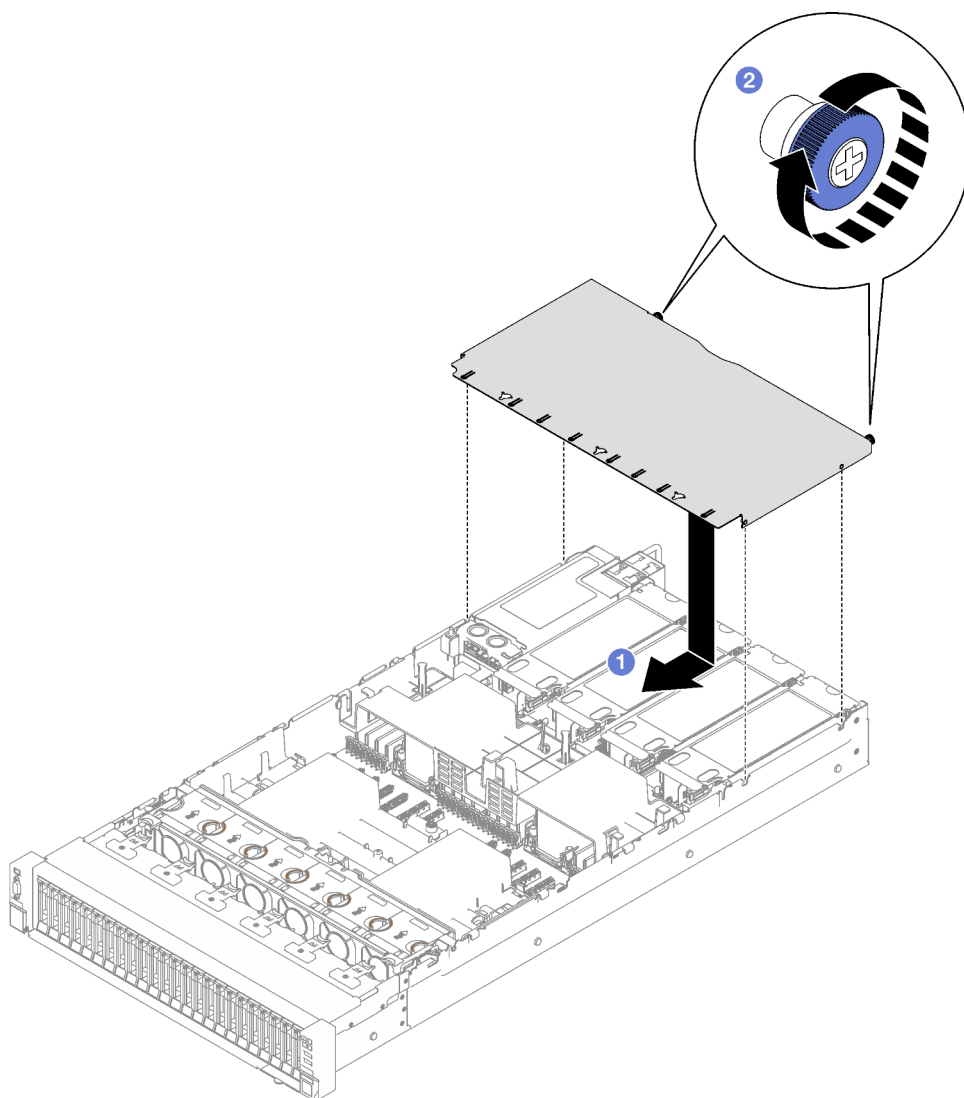
Figura 139. Instalación de la cubierta superior posterior
