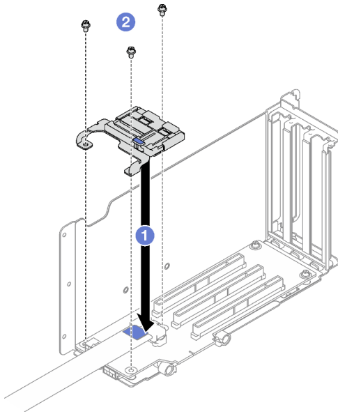
Figura 97. Instalación del elemento de sujeción de PCIe
