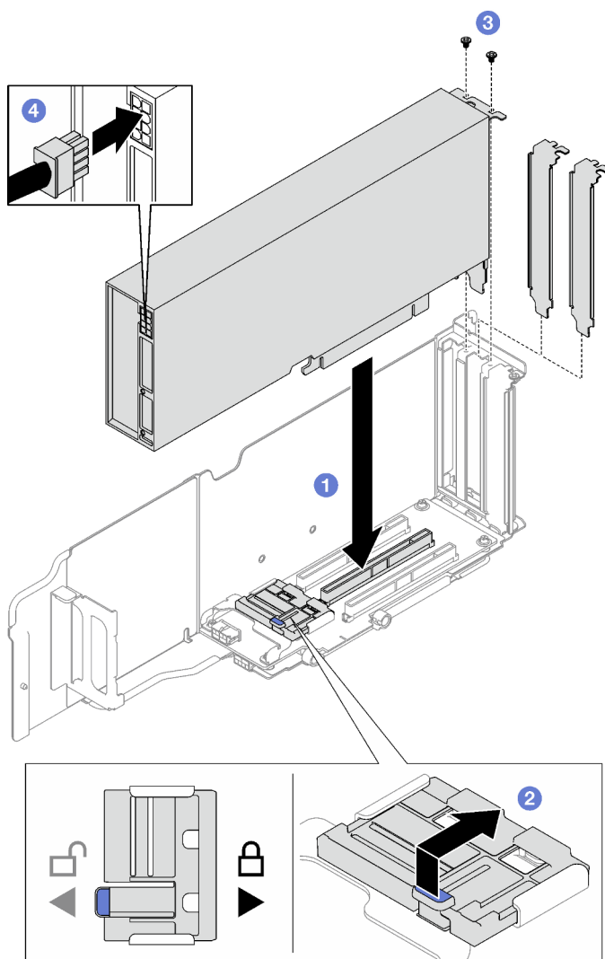
Figura 50. Instalación de un adaptador de GPU de ancho doble
