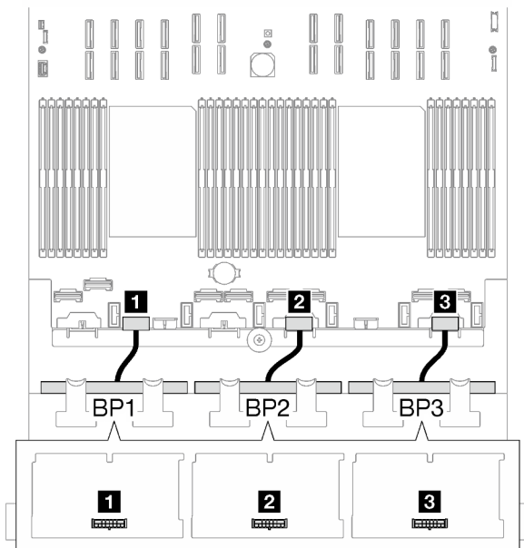
Figura 151. Disposición de los cables de alimentación para las placas posteriores de una unidad de 2,5 pulgadas
