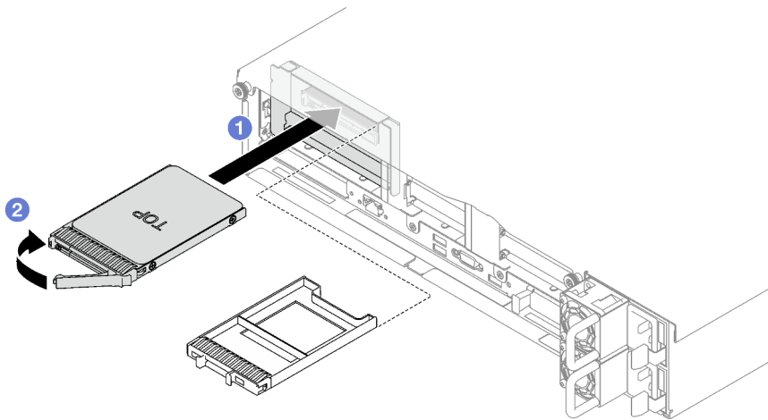
Figura 13. Instalación de la unidad de 7 mm
