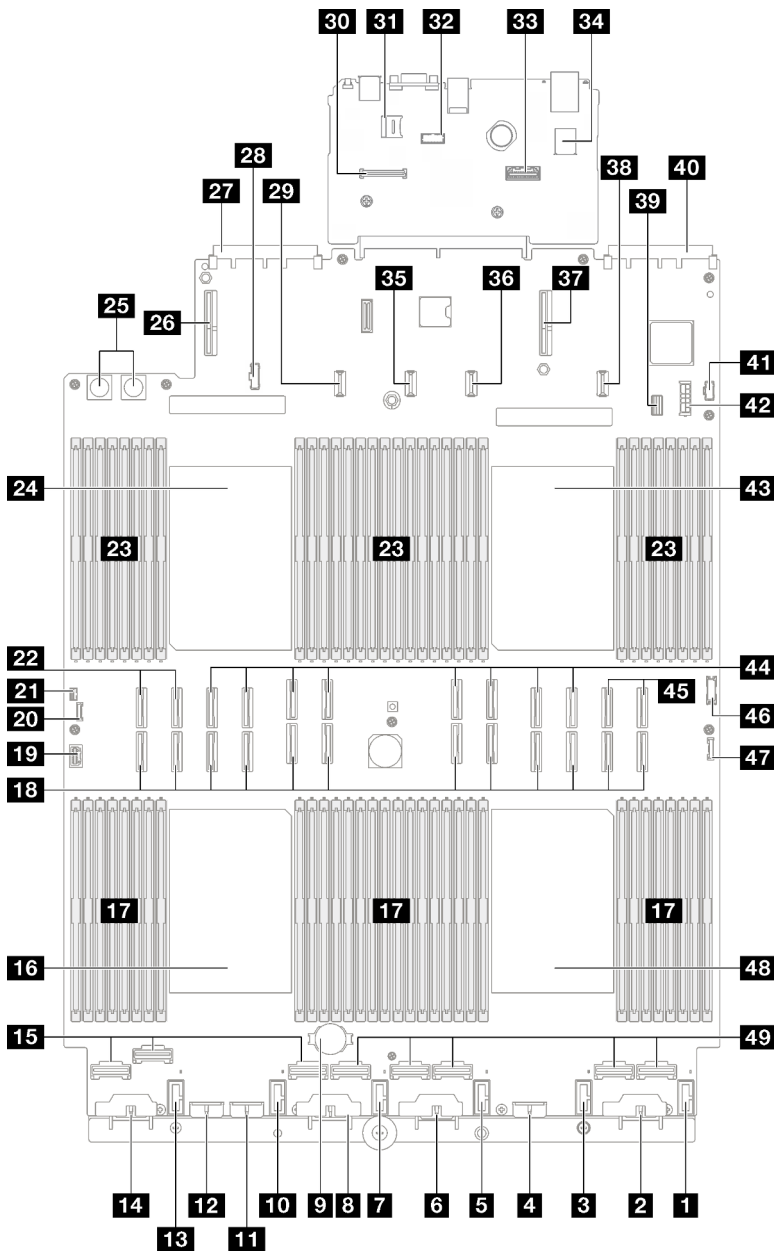
Figura 150. Conectores del conjunto de la placa del sistema
