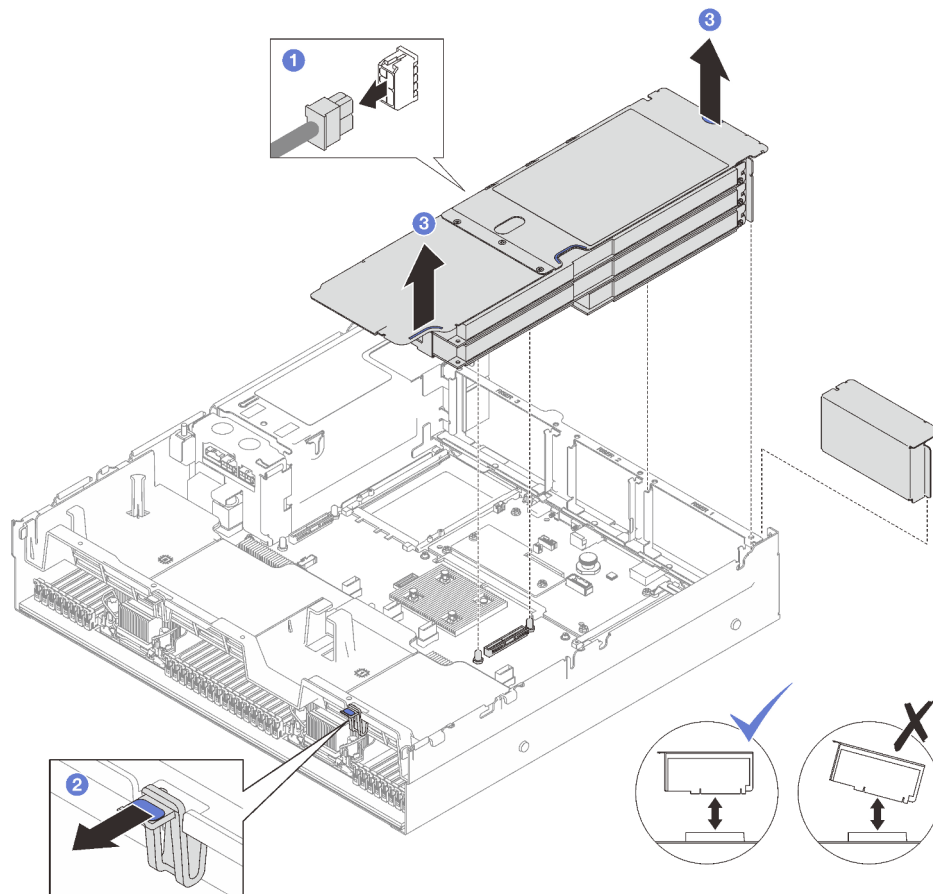
Figura 76. Extracción de una expansión PCIe de FHFL
