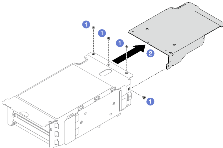
Figura 98. Extracción del amplificador de expansión PCIe
