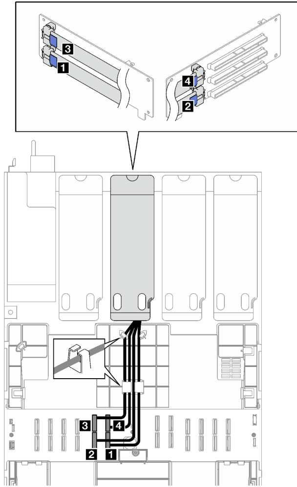
Figura 171. Disposición de cables para la expansión PCIe C
