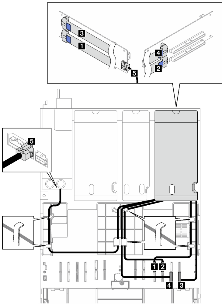
Figura 159. Disposición de cables para la expansión de dos ranuras PCIe de HL 1
