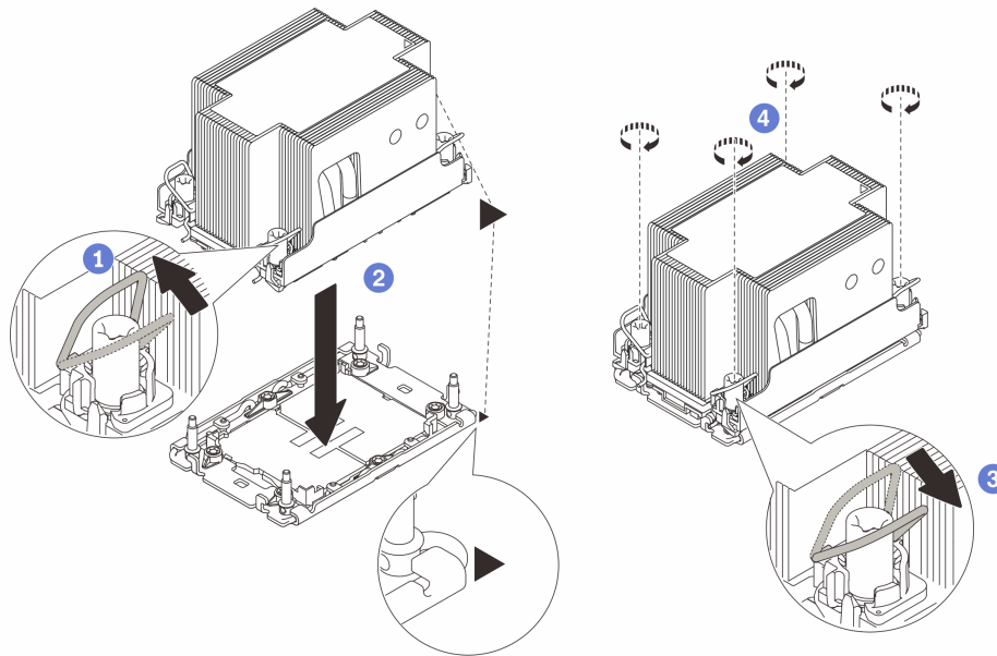
Figura 118. Instalación de PHM estándar 2U
