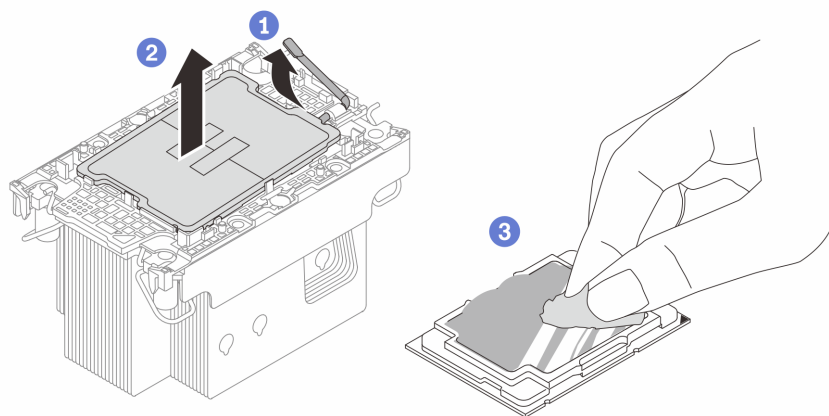
Figura 112. Separación de un procesador del disipador de calor y del transportador
