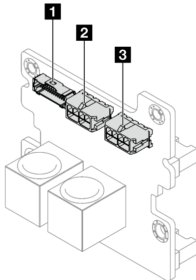
Figura 149. Conectores de placa de distribución de alimentación
