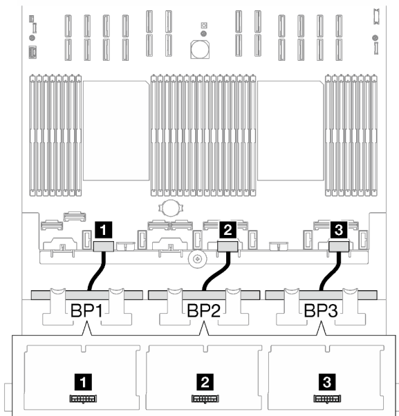
Figura 152. Disposición de los cables de alimentación para las placas posteriores de una unidad de 2,5 pulgadas
