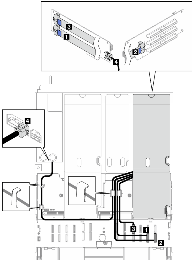
Figura 164. Disposición de cables para la expansión de tres ranuras PCIe de FL 1
