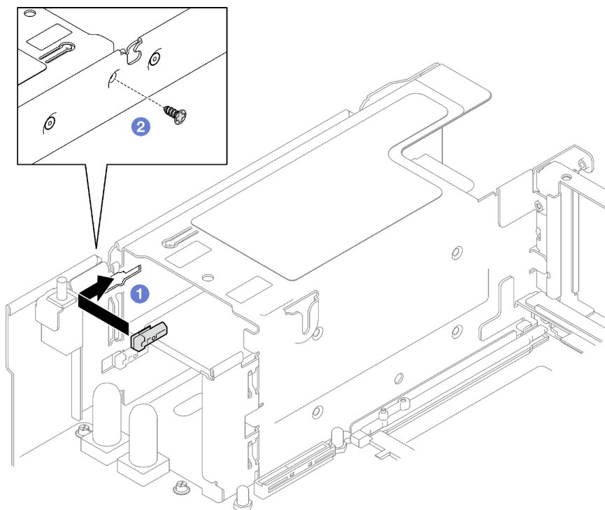
Figura 108. Instalación de una llave de fuente de alimentación
