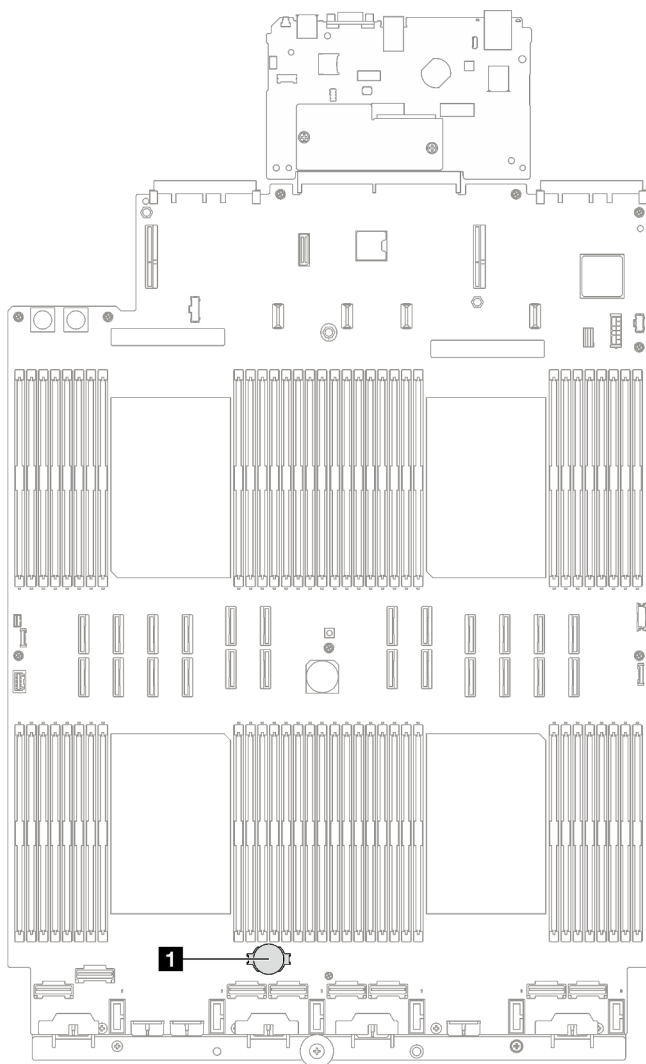
Figura 30. Ubicación de batería CMOS
