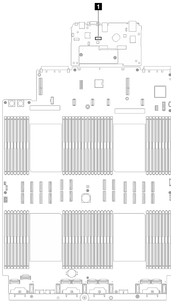
Figura 128. Ubicación del conector del puerto serie
