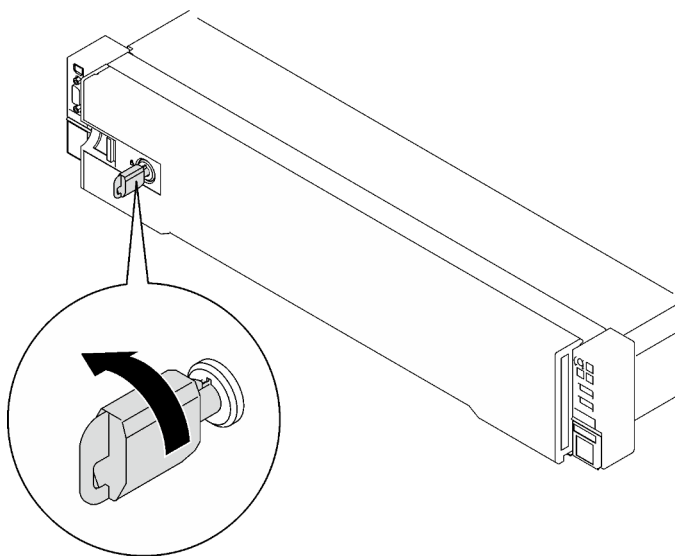
Figura 125. Bloqueo del marco biselado de seguridad
