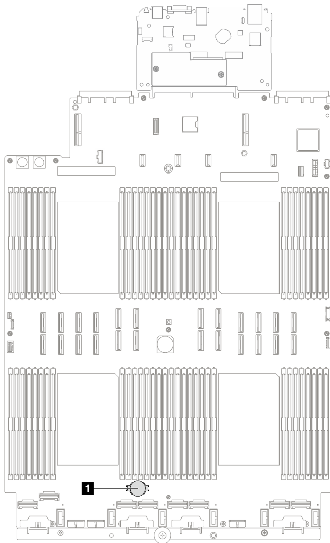
Figura 33. Ubicación del zócalo de la batería CMOS
