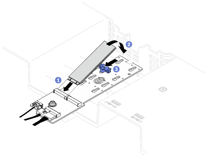
Figura 62. Instalación de la unidad M.2
