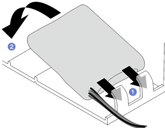
Figura 45. Instalación del módulo de alimentación flash
