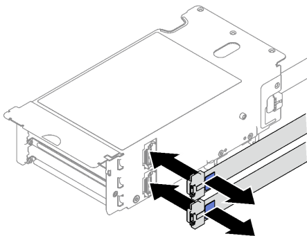
Figura 93. Conexión de cable
