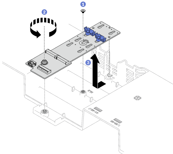
Figura 54. Extracción de la placa posterior M.2
