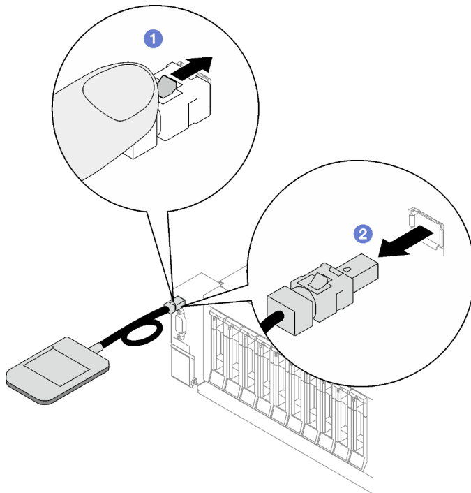
Figura 35. Desconexión del cable del auricular de diagnóstico externo
