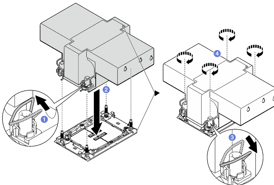
Figura 119. Instalación de PHM de rendimiento 2U
