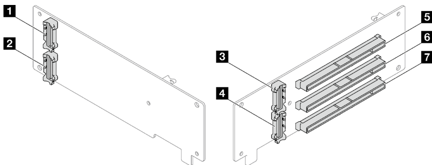
Figura 147. Conectores de la tarjeta de expansión de tres ranuras PCIe Gen4 (sin conector de alimentación)
