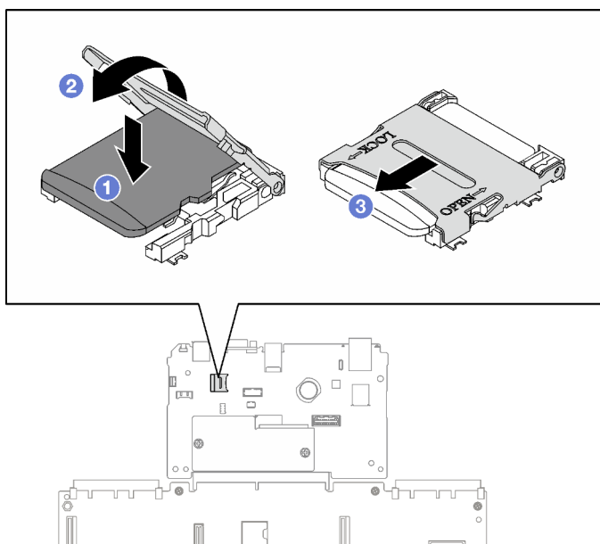
Figura 70. Tarjeta microSD, instalación
