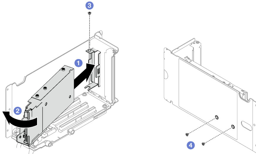
Figura 12. Instalación de compartimiento de la unidad de 7 mm
