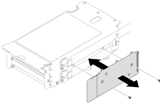
Figura 94. Instalación de la cubierta de cable
