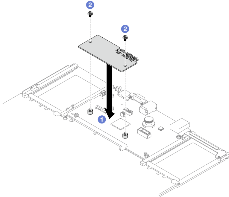
Figura 131. Instalación del Firmware y módulo de seguridad de RoT
