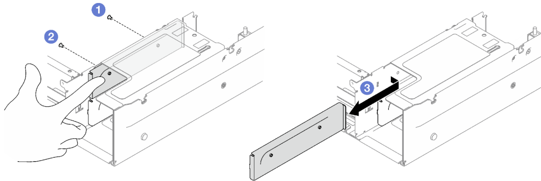
Figura 105. Extracción del soporte de fuente de alimentación
