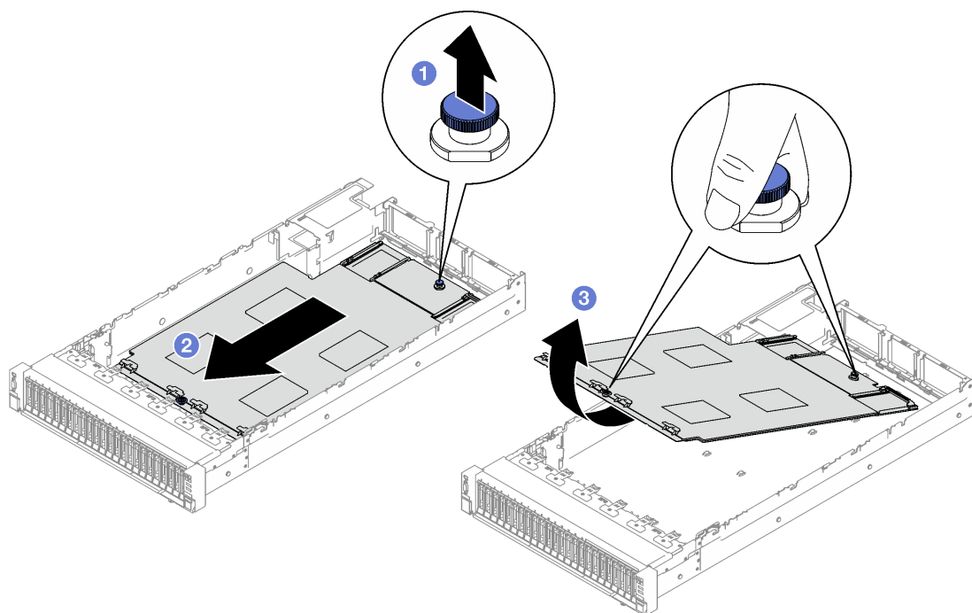
Figura 132. Extracción del conjunto de la placa del sistema
