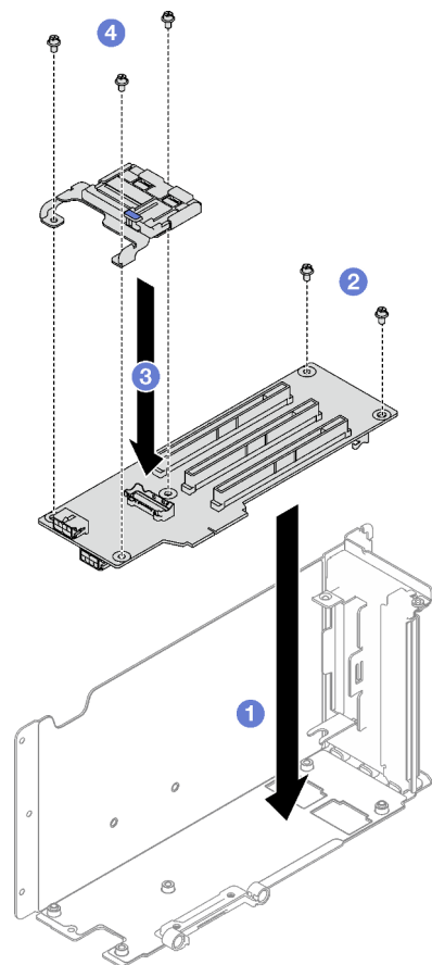
Figura 95. Instalación de la tarjeta de expansión PCIe
