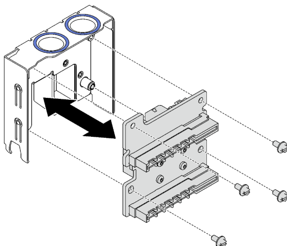
Figura 101. Desensamblaje de la placa de distribución de alimentación
