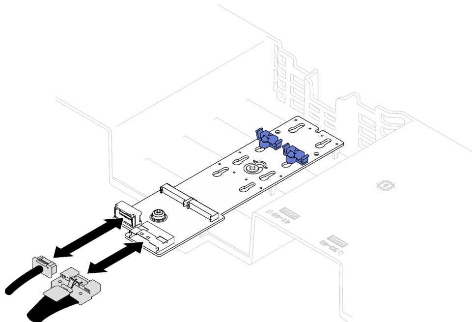
Figura 16. Desconexión de cable de la placa posterior SATA/x4 NVMe M.2
