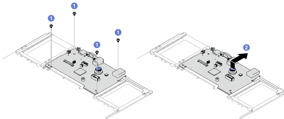
Figura 133. Extracción de la placa de E/S del sistema
