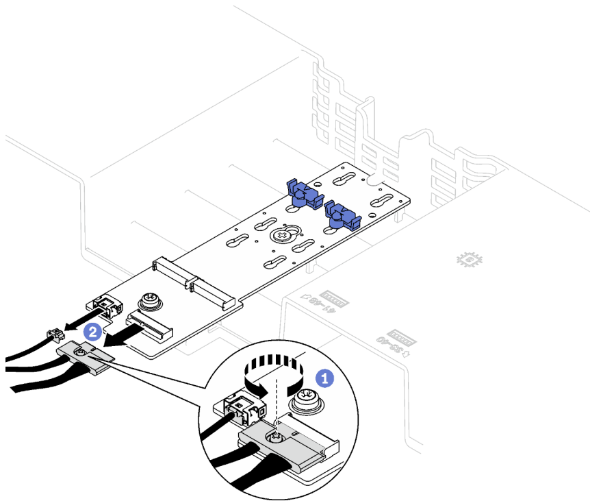
Figura 23. Desconexión de cable de la placa posterior SATA/NVMe M.2
