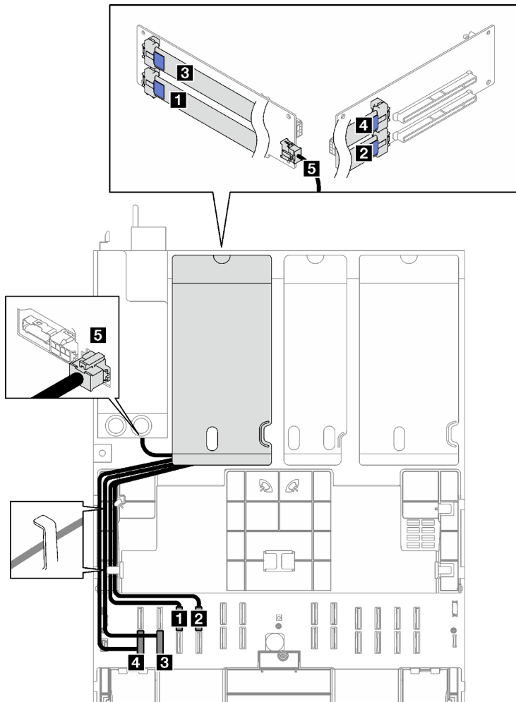
Figura 167. Disposición de cables para la expansión de dos ranuras PCIe 3
