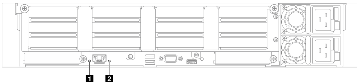
Figura 182. LED de sistema en la vista posterior: modelo de servidor con cuatro expansiones PCIe
