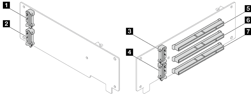
Figura 148. Conectores de la tarjeta de expansión de tres ranuras PCIe Gen5 (sin conector de alimentación)
