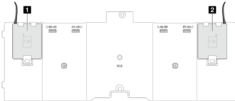
Figura 44. Ubicación de la ranura del módulo de alimentación flash
