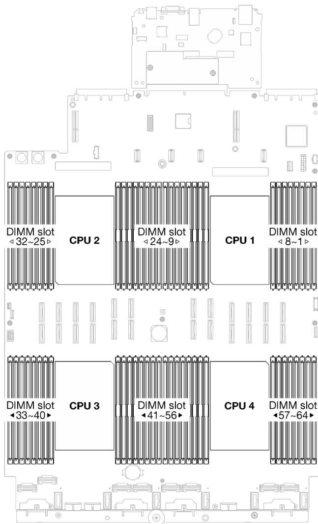
Figura 65. Diseño de los módulos de memoria y el procesador
