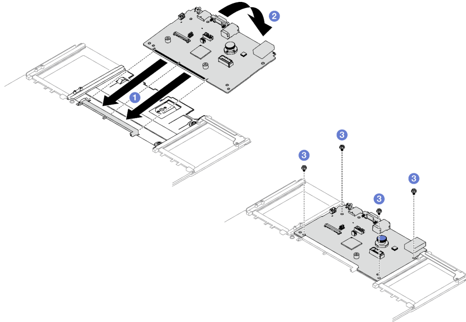
Figura 134. Instalación de la placa de E/S del sistema
