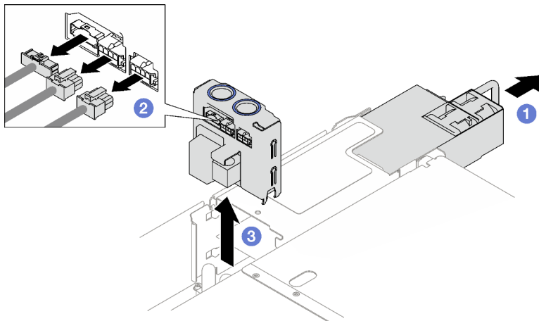
Figura 100. Extracción de la placa de distribución de alimentación
