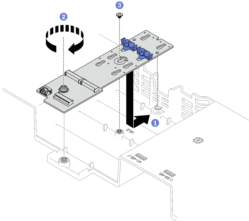
Figura 59. Instalación de la placa posterior M.2
