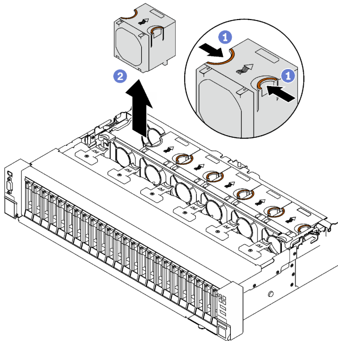
Figura 38. Extracción del ventilador
