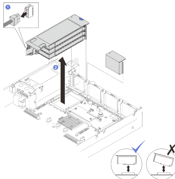
Figura 74. Extracción de la expansión PCIe de LP (con conector de alimentación)
