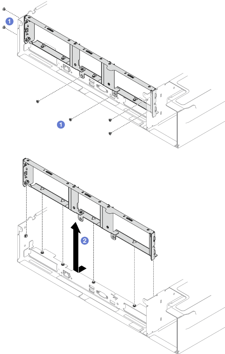
Figura 120. Extracción de la pared posterior
