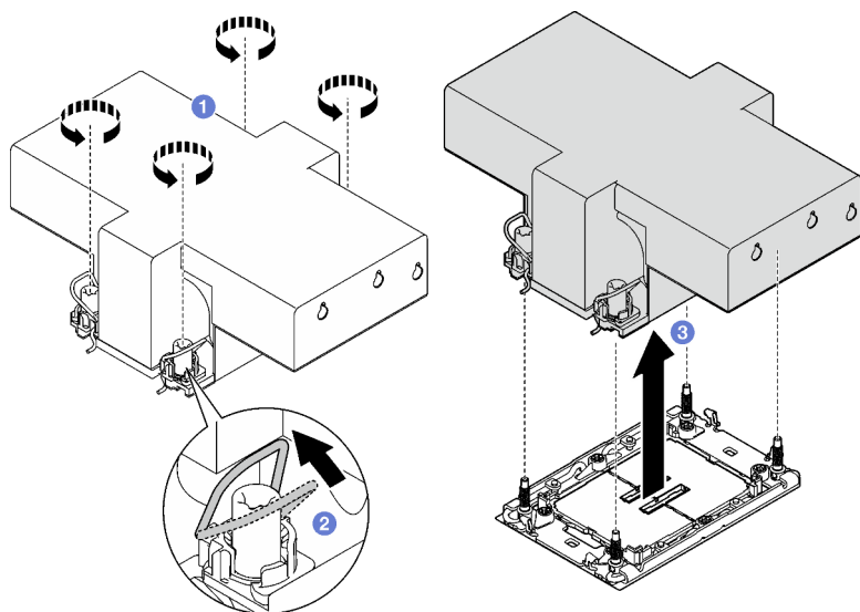
Figura 111. Extracción de PHM de rendimiento 2U
