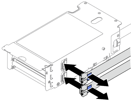
Figura 86. Desconexión de cable
