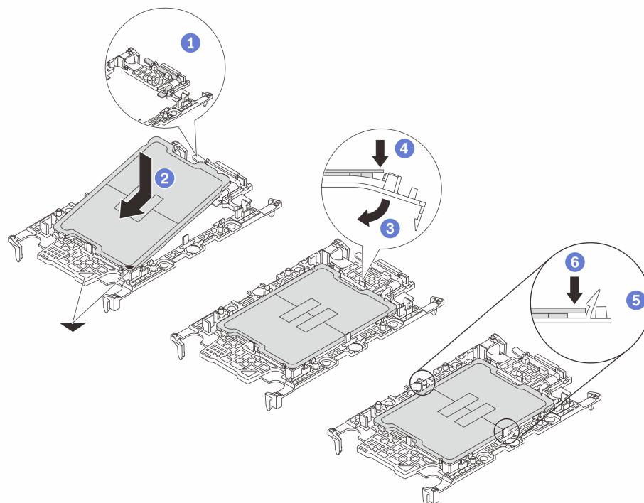
Figura 115. Instalación del transportador del procesador
