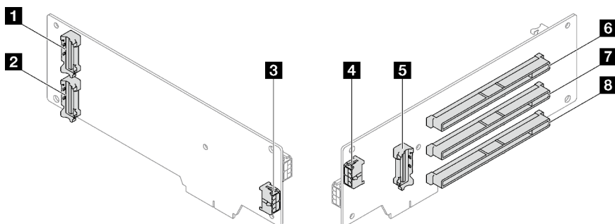
Figura 146. Conectores de la tarjeta de expansión de tres ranuras PCIe Gen5 (con conector de alimentación)
