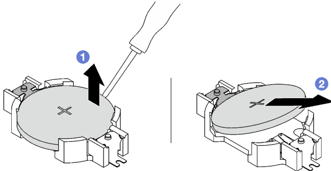
Figura 32. Extracción de la batería CMOS
