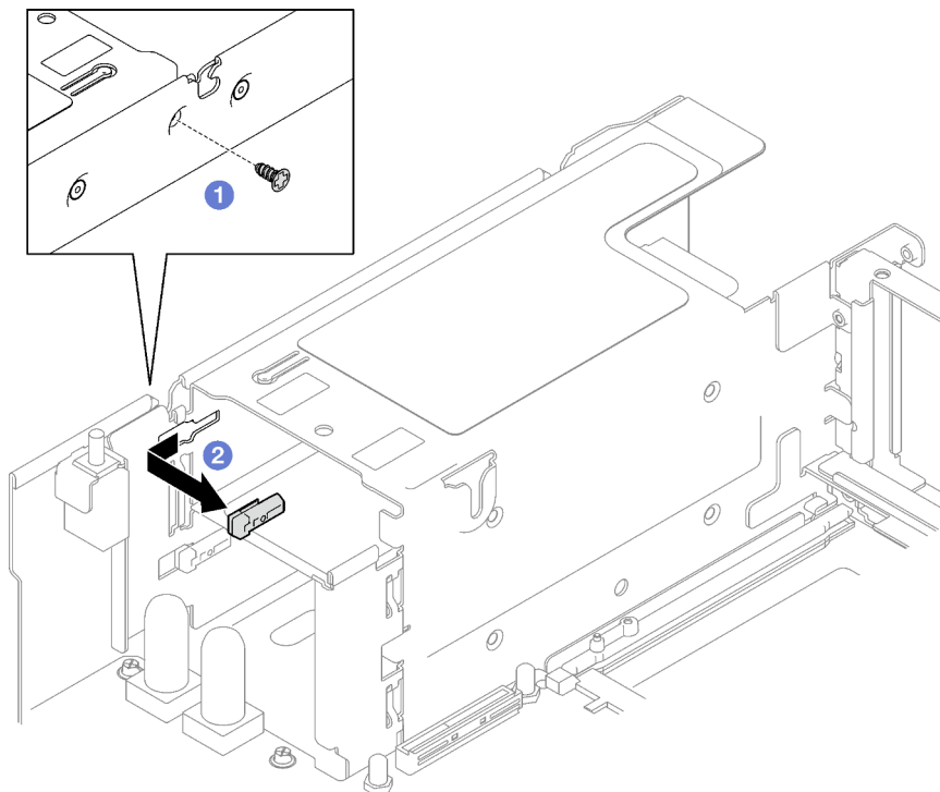
Figura 107. Extracción de la llave de fuente de alimentación
