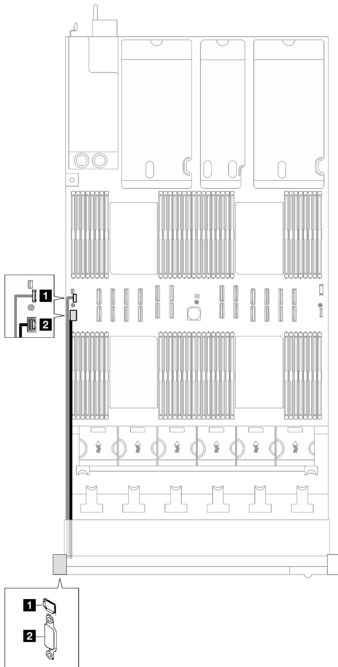
Figura 153. Disposición de cables para el auricular de diagnóstico externo y la VGA
