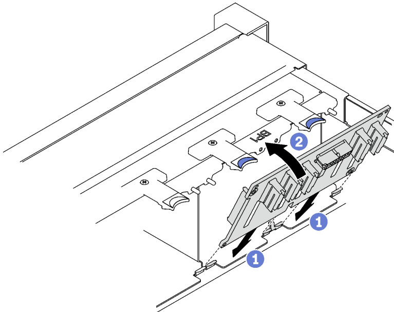
Figura 6. Instalación de la placa posterior de la unidad de 2,5 pulgadas
