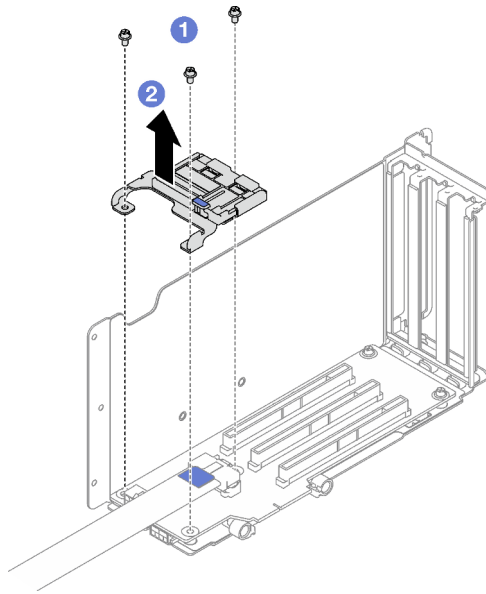
Figura 96. Extracción del elemento de sujeción de PCIe
