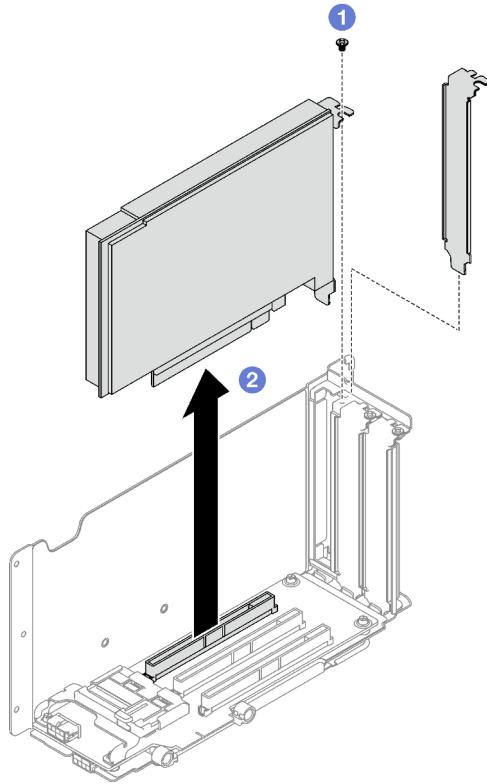
Figura 77. Extracción del adaptador PCIe
