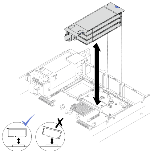
Figura 73. Extracción de la expansión PCIe de LP (sin conector de alimentación)
