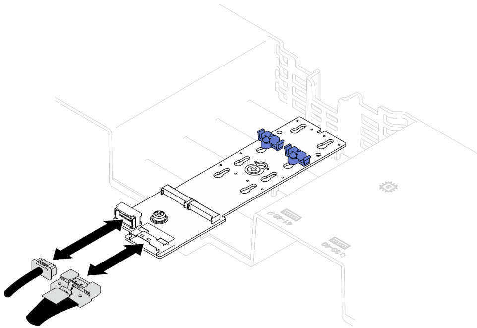
Figura 24. Desconexión de cable de la placa posterior SATA/x4 NVMe M.2
