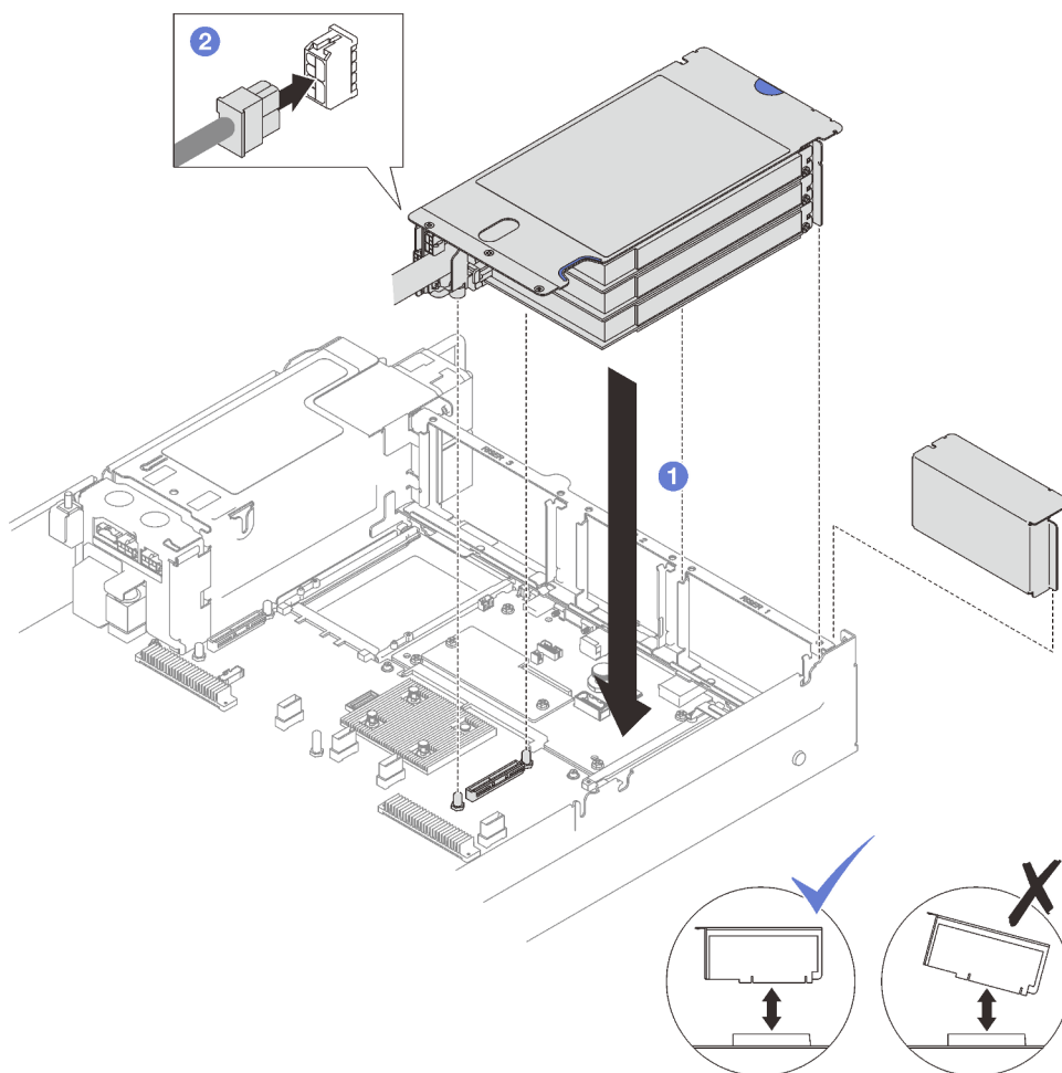
Figura 83. Instalación de expansión PCIe de FHHL
