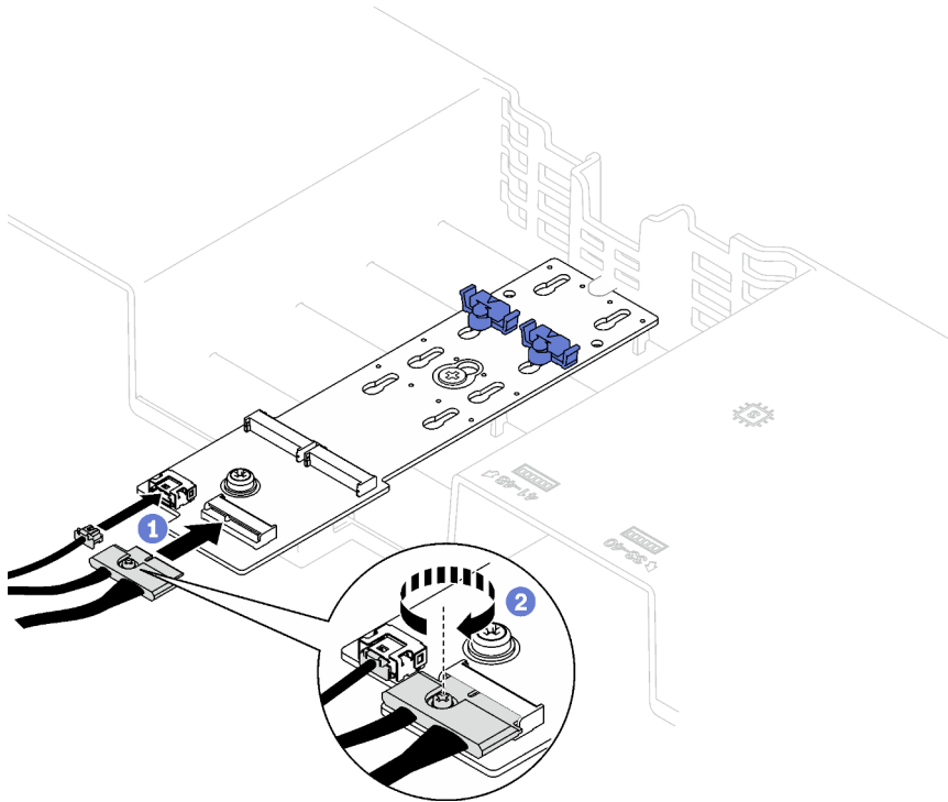
Figura 27. Conexión de cable de la placa posterior SATA/NVMe M.2
