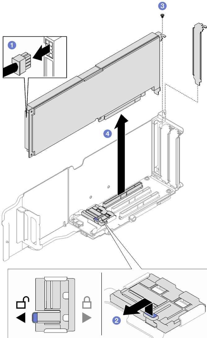
Figura 47. Extracción un adaptador de GPU de ancho único
