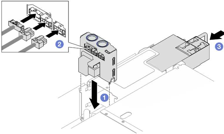
Figura 102. Instalación de la placa de distribución de alimentación
