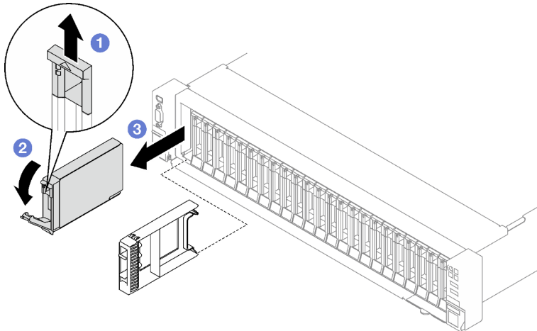
Figura 3. Extracción de la unidad de intercambio en caliente de 2,5 pulgadas
