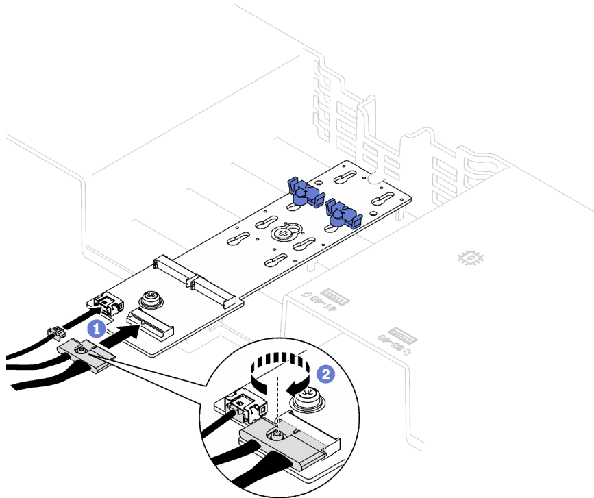
Figura 57. Conexión del cable de la placa posterior M.2 SATA/NVMe o NVMe
