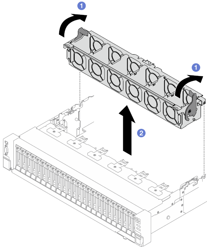
Figura 39. Extracción de la caja del ventilador
