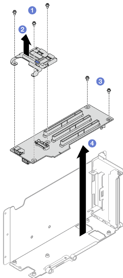
Figura 88. Extracción de tarjeta de expansión PCIe
