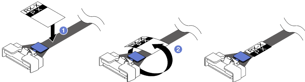
Figura 90. Aplicación de la etiqueta
