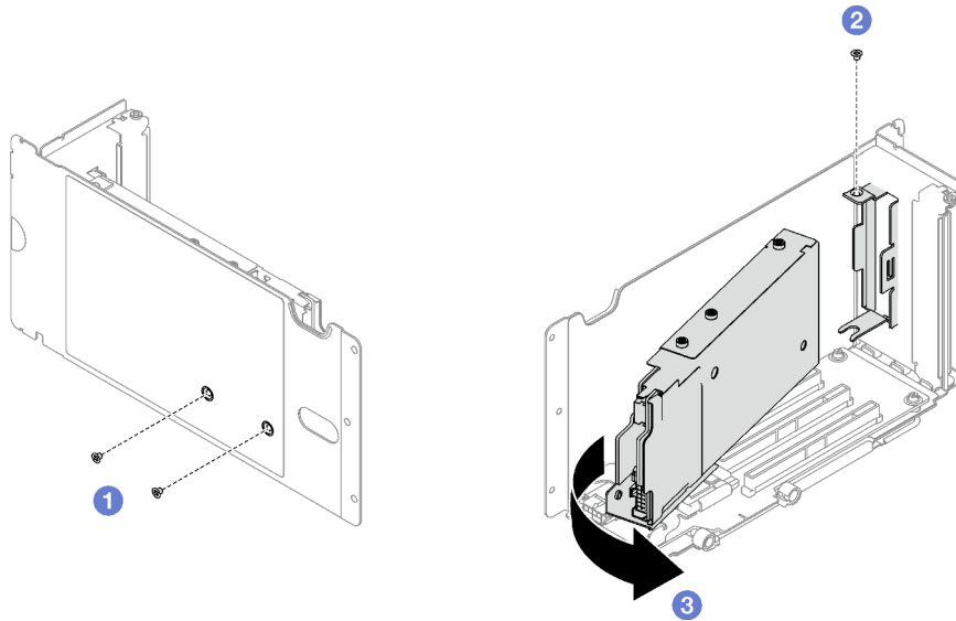
Figura 9. Extracción del compartimiento de la unidad de 7 mm
