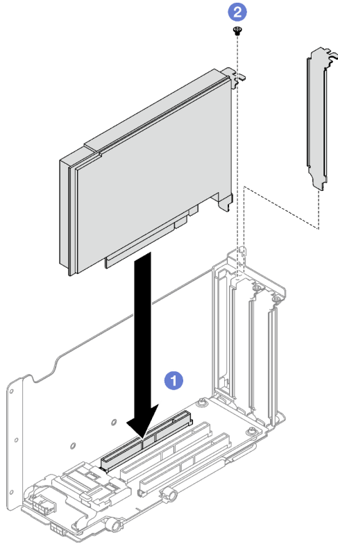
Figura 78. Instalación de adaptador PCIe
