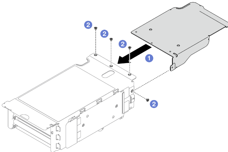
Figura 99. Instalación del amplificador de expansión PCIe
