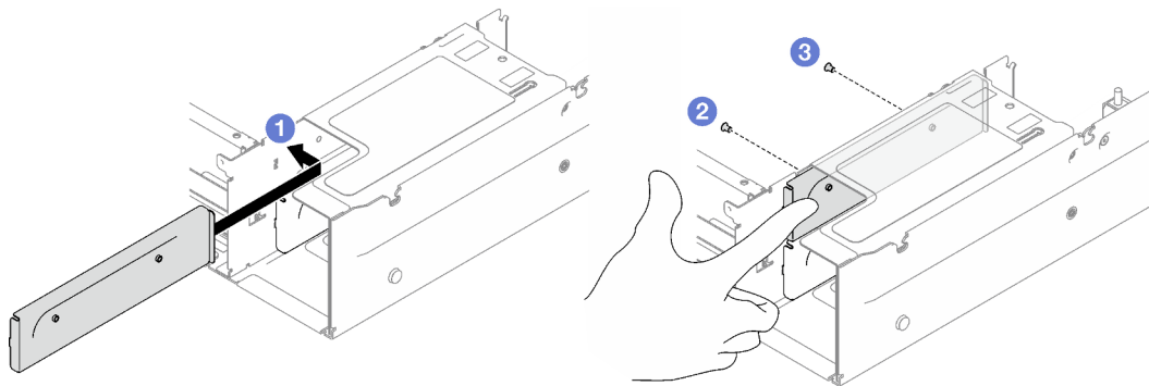
Figura 106. Instalación de un soporte de fuente de alimentación
