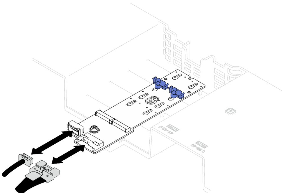
Figura 56. Desconexión de cable de la placa posterior SATA/x4 NVMe M.2
