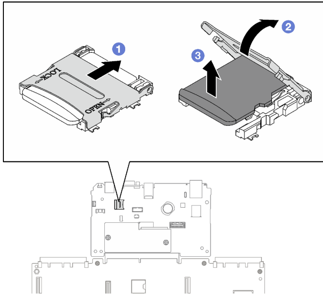
Figura 69. Extracción de la tarjeta microSD
