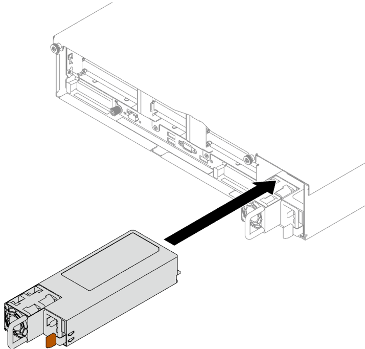
Figura 104. Instalación de la unidad de fuente de alimentación
