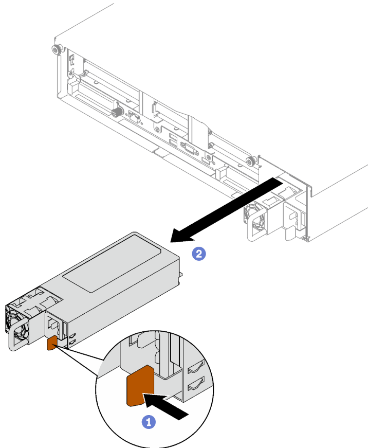
Figura 103. Extracción de la unidad de fuente de alimentación
