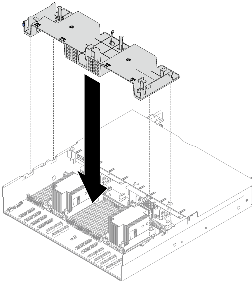
Figura 26. Instalación del deflector de aire posterior
