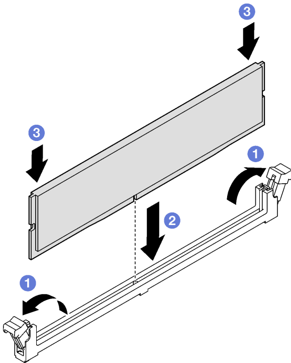
Figura 68. Instalación de un módulo de memoria
