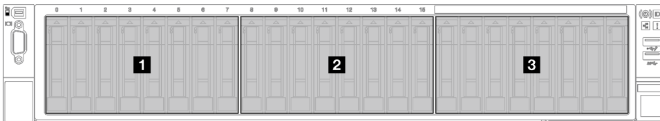
Figura 5. Numeración de la placa posterior de unidad de 2,5 pulgadas
