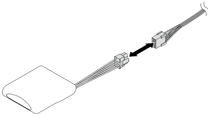
Figura 42. Desconexión del cable del módulo de alimentación flash
