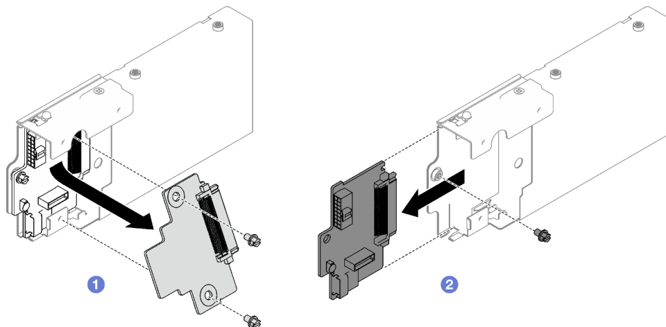
Figura 10. Extracción de la placa posterior de la unidad de 7 mm
