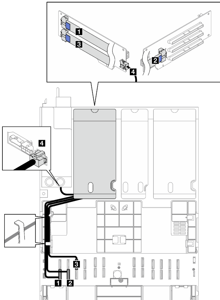
Figura 168. Disposición de cables para la expansión de tres ranuras PCIe 3
