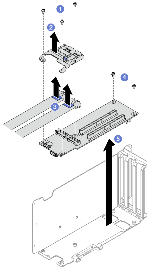
Figura 87. Extracción de tarjeta de expansión PCIe
