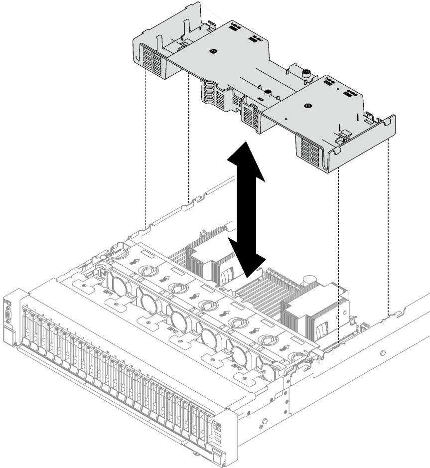
Figura 18. Instalación del deflector de aire frontal
