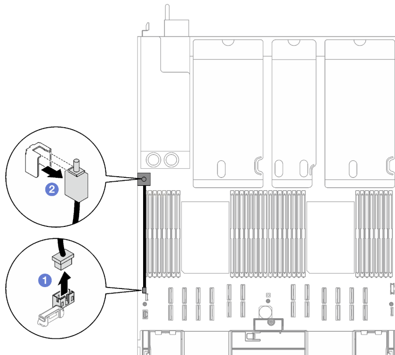
Figura 51. Extracción del conmutador de intrusión
