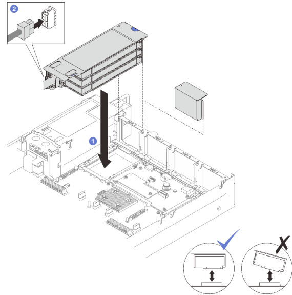
Figura 82. Instalación de la expansión PCIe de LP (con conector de alimentación)
