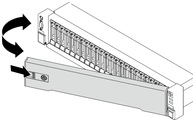
Figura 124. Instalación del marco biselado de seguridad
