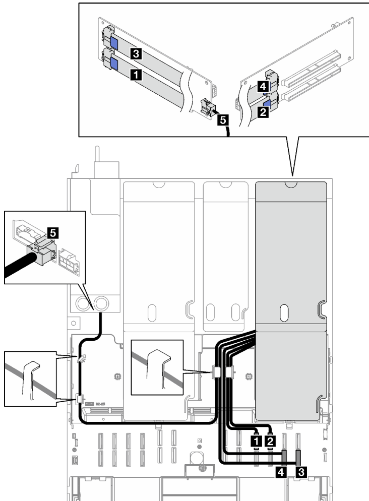
Figura 160. Disposición de cables para la expansión de dos ranuras PCIe de FL 1
