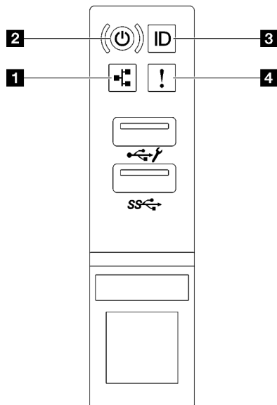
Figura 178. LED del módulo de E/S frontal
