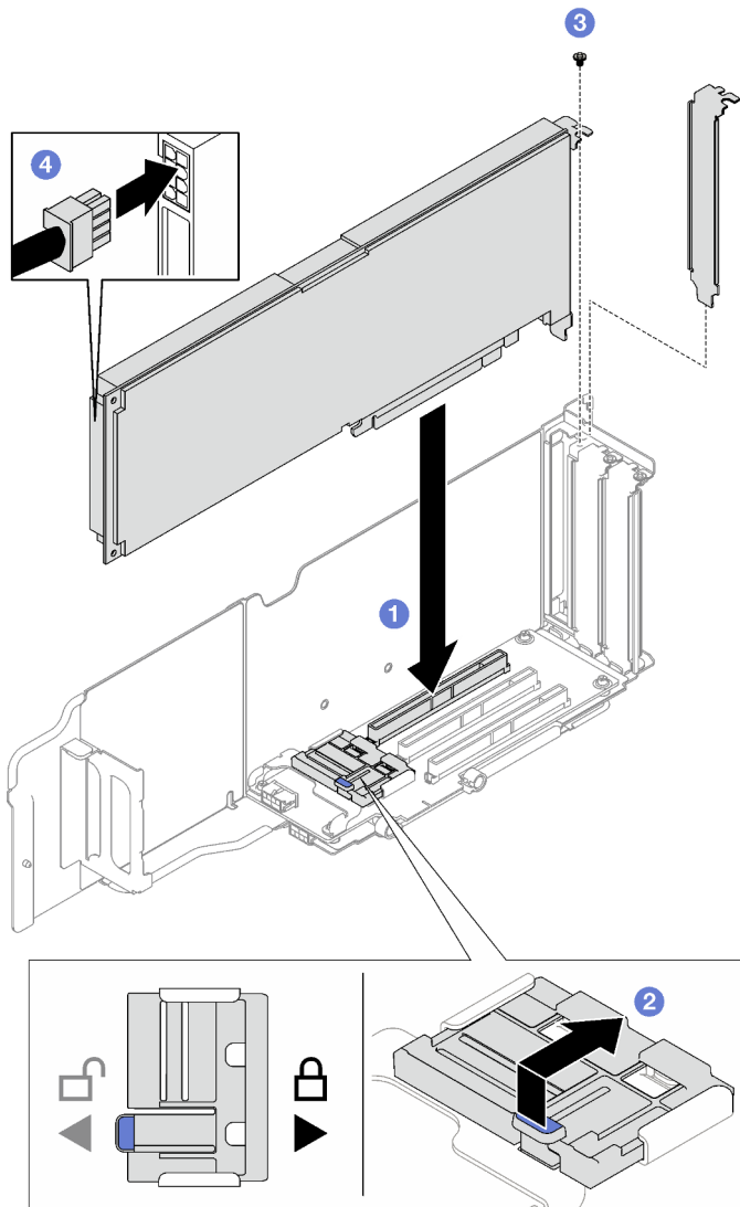
Figura 49. Instalación de un adaptador de GPU de ancho único
