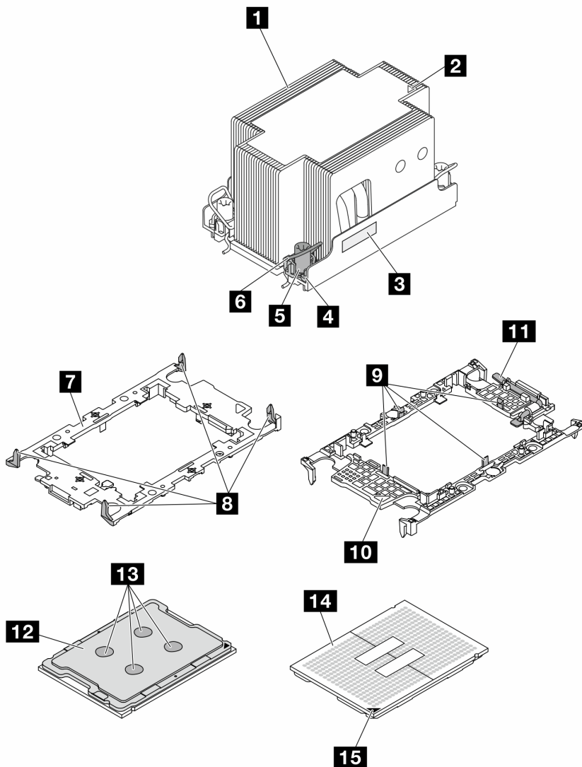
Figura 114. Componentes de PHM
