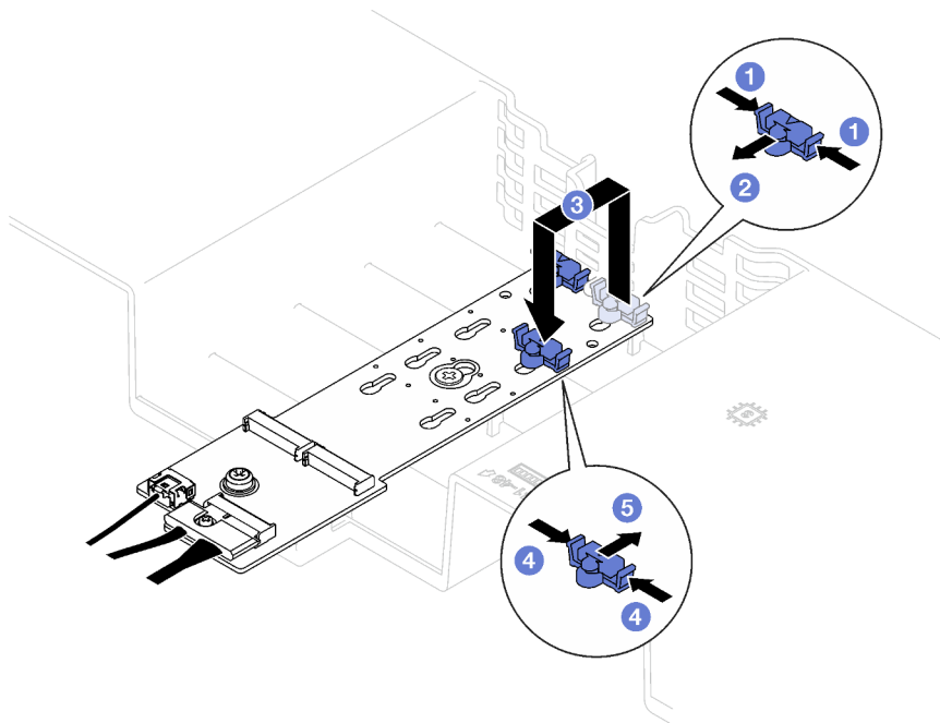
Figura 60. Ajuste del elemento de sujeción de la placa posterior de M.2
