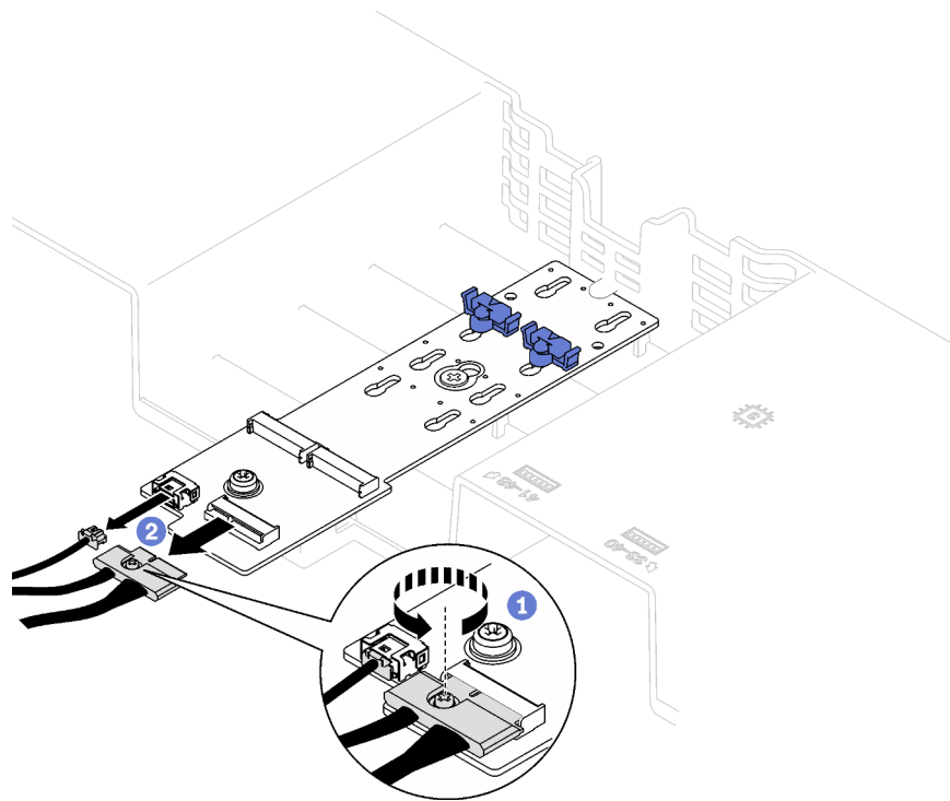
Figura 15. Desconexión de cable de la placa posterior SATA/NVMe M.2
