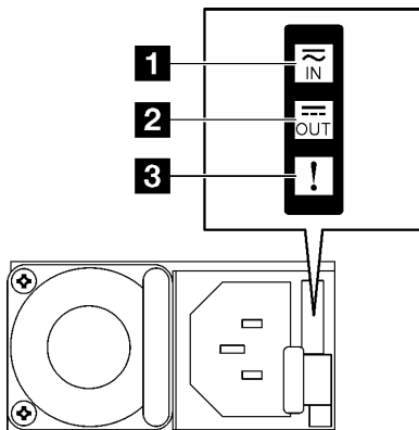
Figura 179. LED de fuente de alimentación CFFv4
