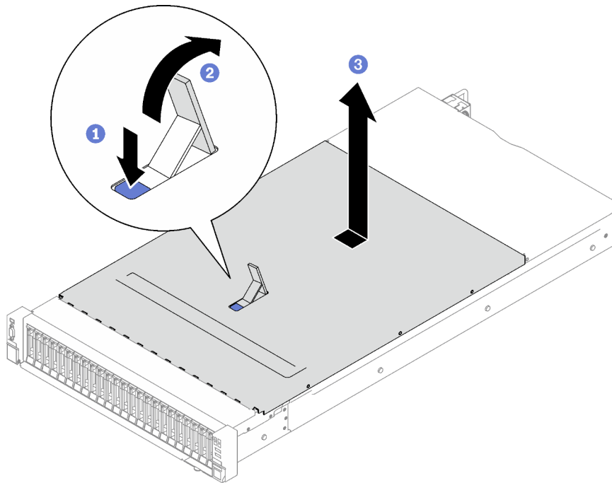
Figura 137. Extracción de la cubierta superior frontal
