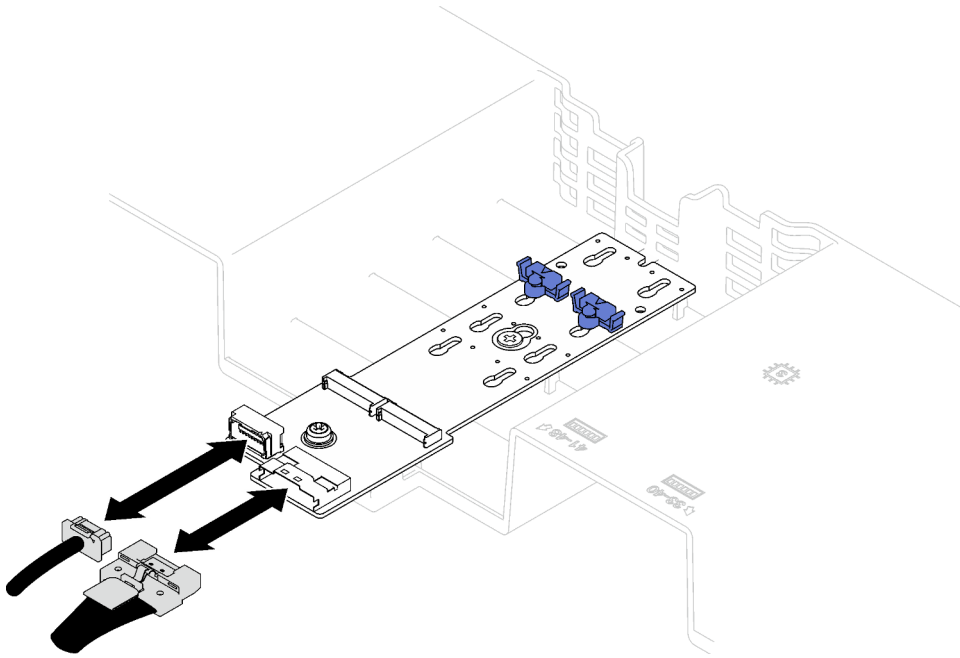
Figura 58. Conexión de cable de la placa posterior SATA/x4 NVMe M.2
