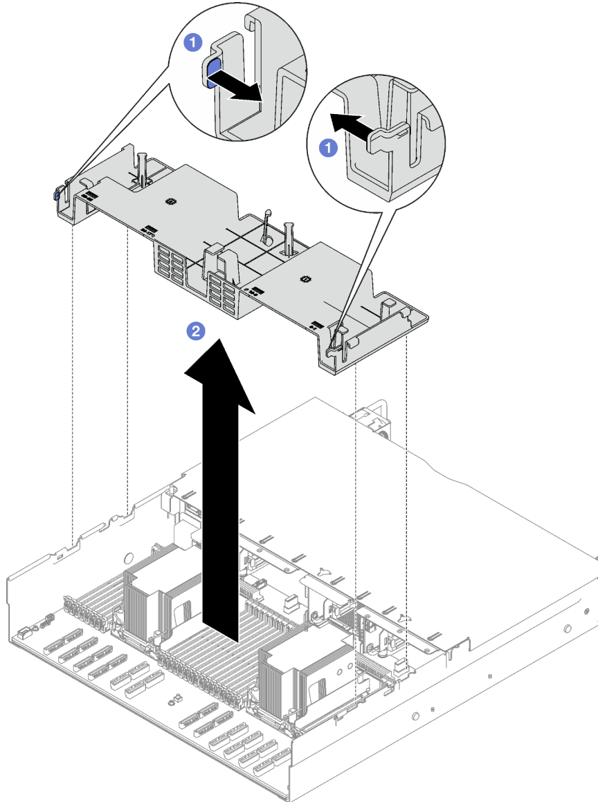
Figura 25. Extracción del deflector de aire posterior
