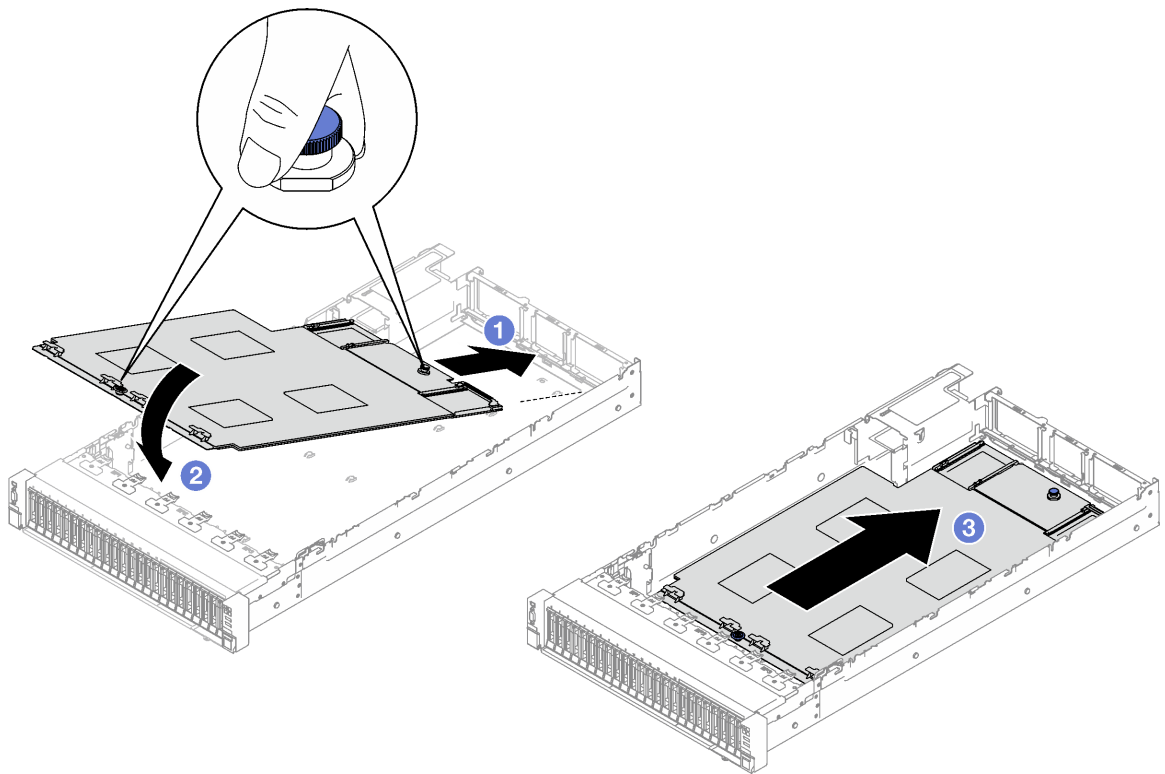
Figura 135. Instalación del conjunto de la placa del sistema
