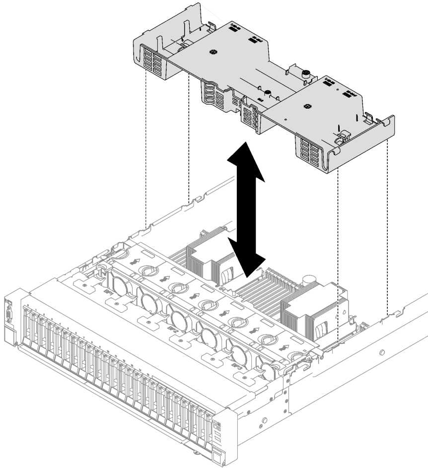
Figura 17. Extracción del deflector de aire frontal
