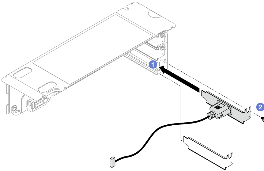
Figura 127. Instalación de módulo de puerto serie
