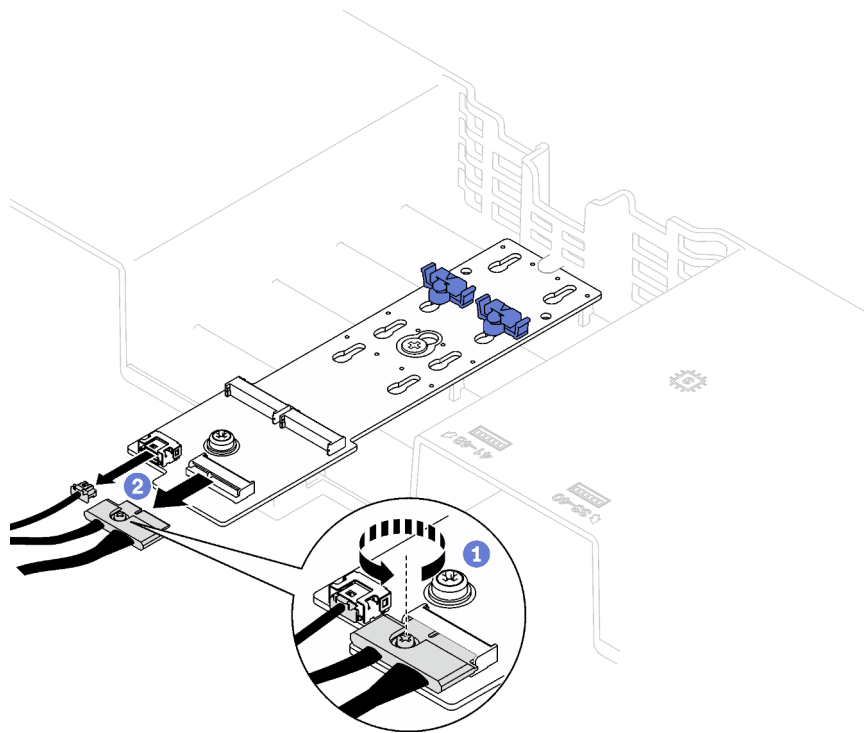
Figura 55. Desconexión del cable de la placa posterior M.2 SATA/NVMe o NVMe
