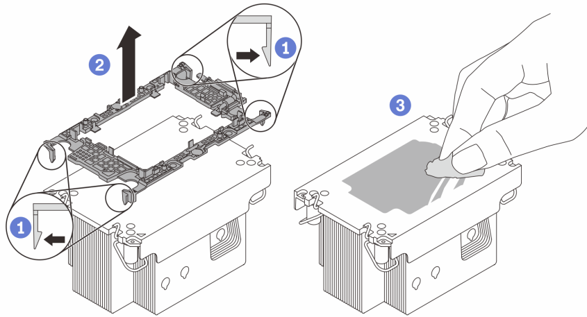
Figura 113. Separación de un transportador de procesador del disipador de calor
