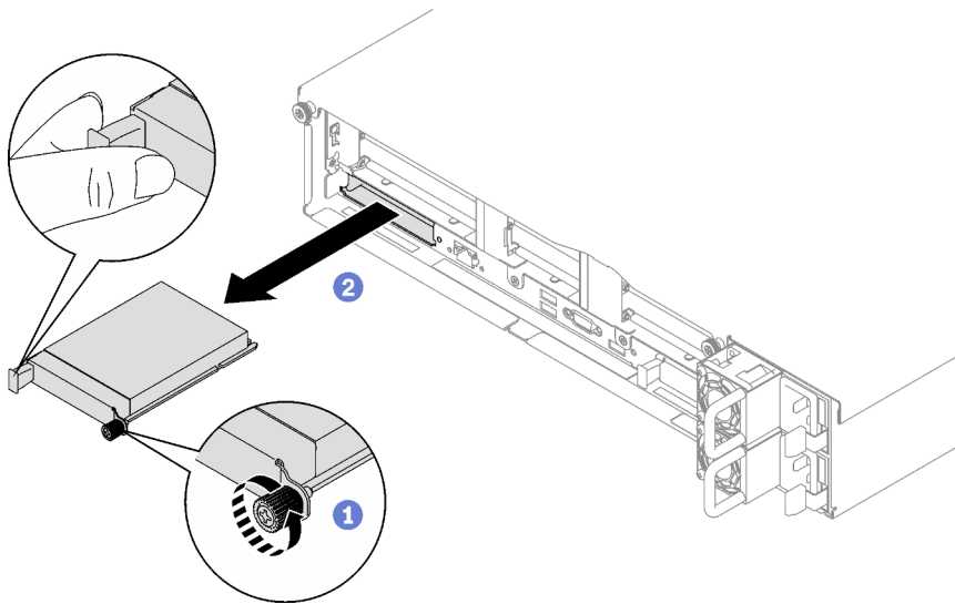
Figura 71. Extracción del módulo de OCP
