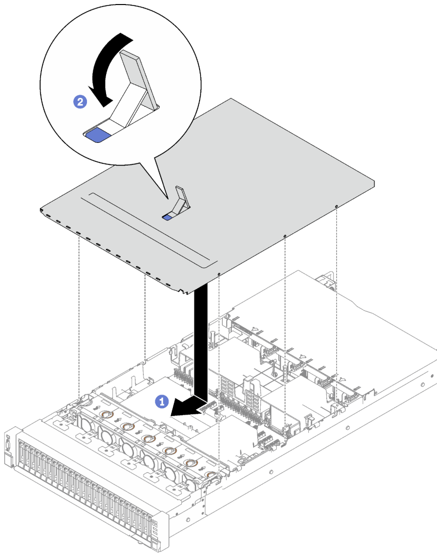
Figura 140. Instalación de la cubierta superior frontal
