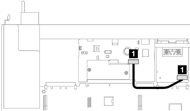
Figura 158. Disposición de los cables adaptador NIC de gestión
