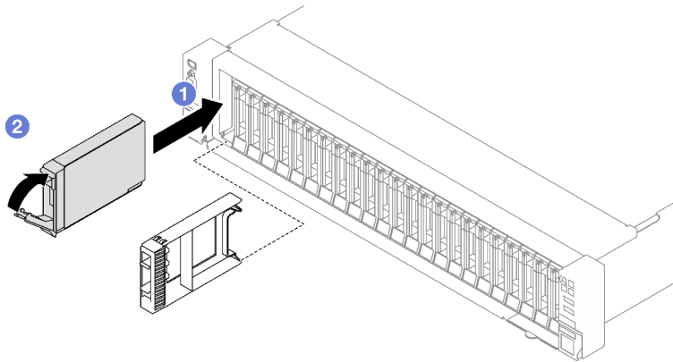
Figura 7. Instalación de unidad de intercambio en caliente de 2,5 pulgadas
