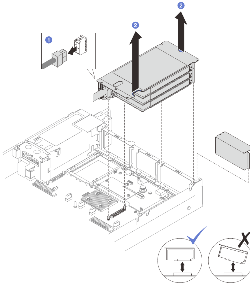
Figura 75. Extracción de una expansión PCIe de FHHL
