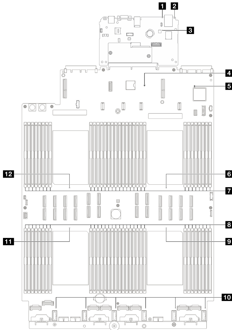
Figura 183. LED del conjunto de la placa del sistema
