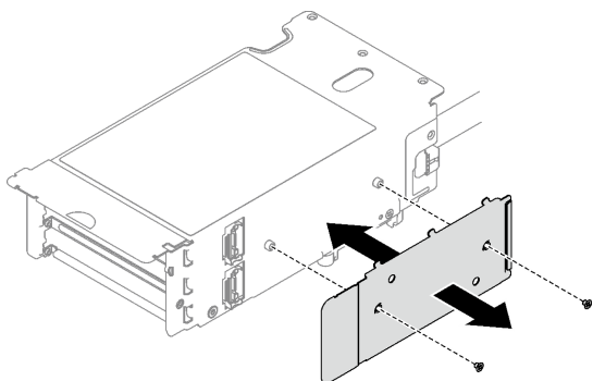
Figura 91. Extracción de la cubierta del cable
