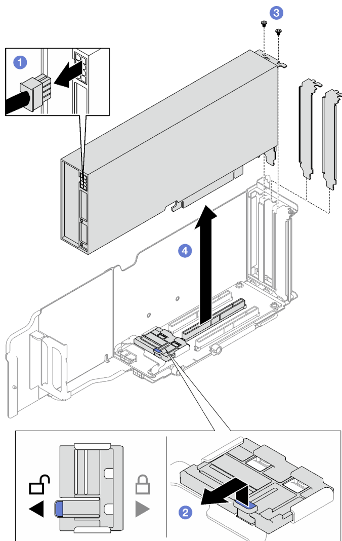
Figura 48. Extracción un adaptador de GPU de ancho doble
