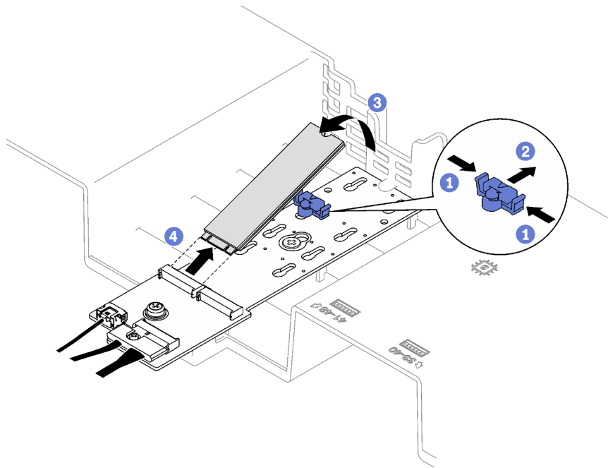
Figura 53. Extracción de la unidad M.2
