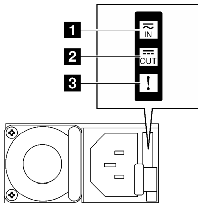
Figura 21. LED de fuente de alimentación CFFv4
