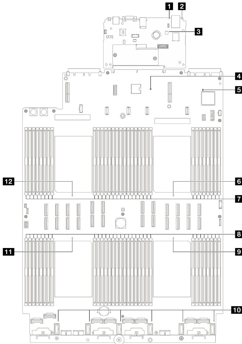
Figura 25. LED del conjunto de la placa del sistema
