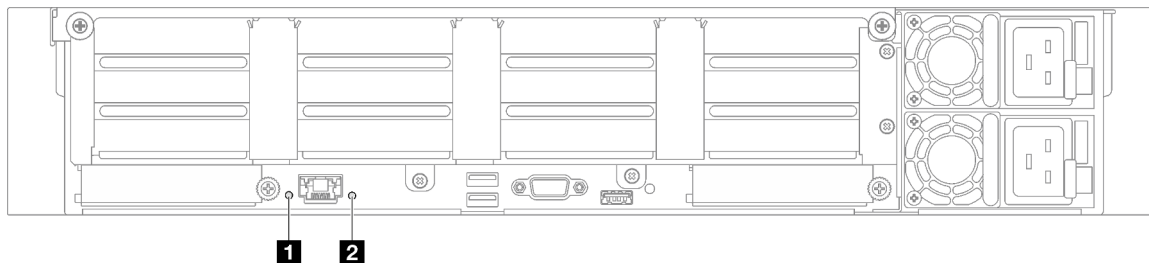
Figura 24. LED de sistema en la vista posterior: modelo de servidor con cuatro expansiones PCIe
