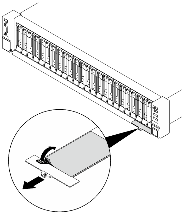
Figura 29. Etiqueta de acceso de red de Lenovo XClarity Controller en la pestaña de información extraíble.
