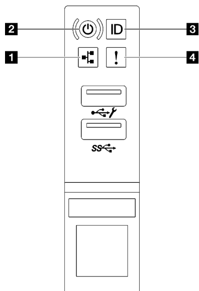
Figura 20. LED del módulo de E/S frontal
