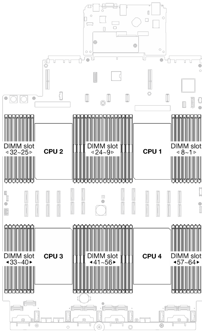
Figure 65. Disposition des modules de mémoire et des processeurs
