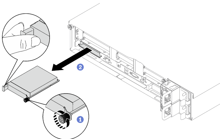
Figure 71. Retrait du module OCP
