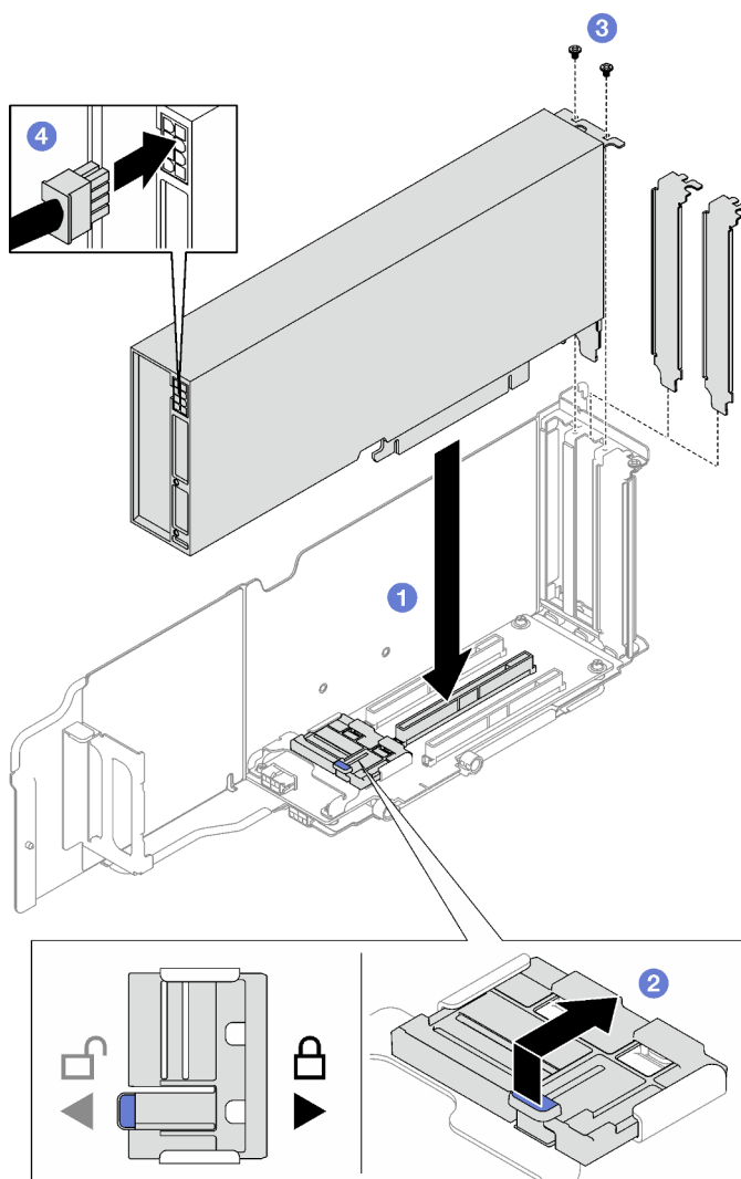
Figure 50. Installation d'un adaptateur GPU double largeur
