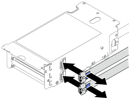
Figure 93. Connexion des câbles
