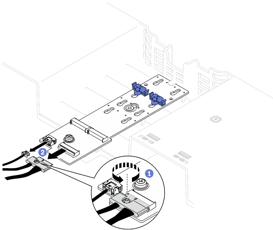
Figure 15. Déconnexion des câbles du fond de panier M.2 SATA/NVMe
