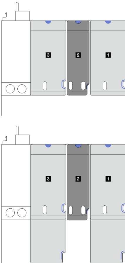
Figure 79. Type et emplacement de carte mezzanine PCIe pour les modèles de serveur dotés de trois cartes mezzanines PCIe
