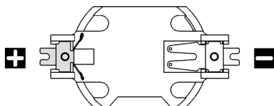
Figure 31. Côté positif (+) et côté (-) de la pile CMOS
