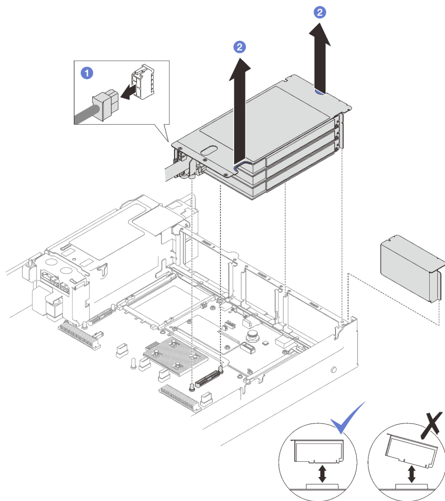
Figure 75. Retrait d'une carte mezzanine PCIe FHHL
