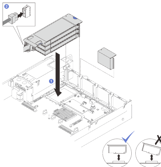
Figure 82. Installation d'une carte mezzanine PCIe LP (avec connecteur d'alimentation)
