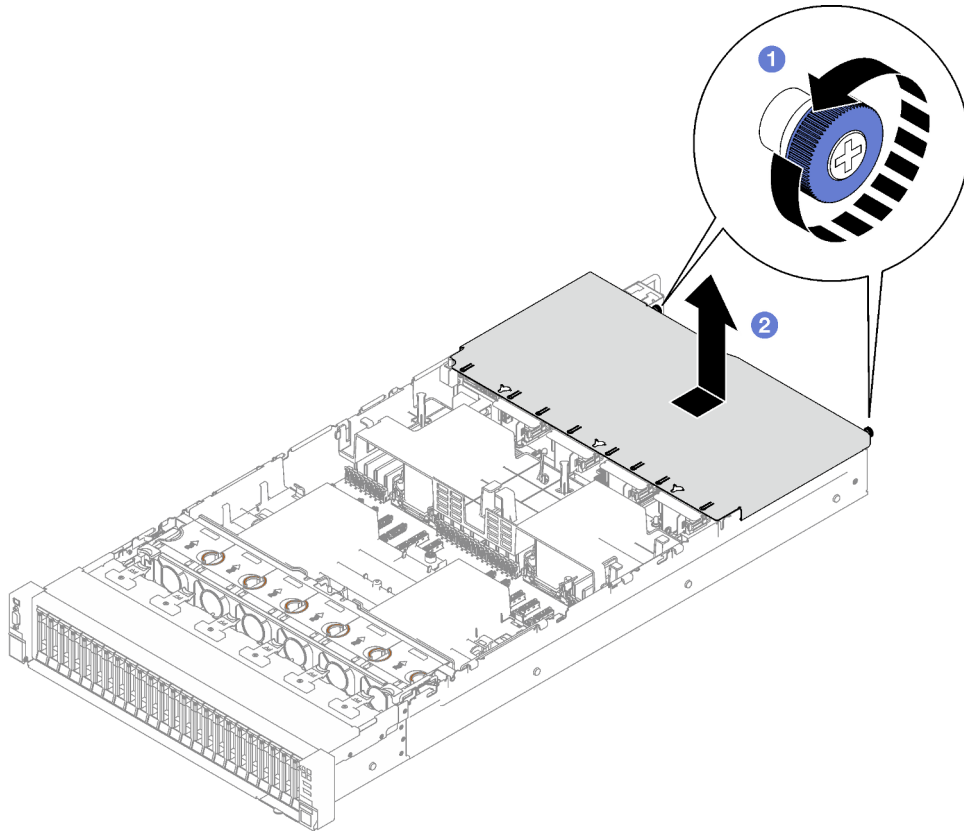
Figure 138. Retrait du carter supérieur arrière
