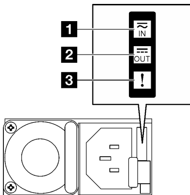
Figure 179. Voyants d'alimentation CFFv4
