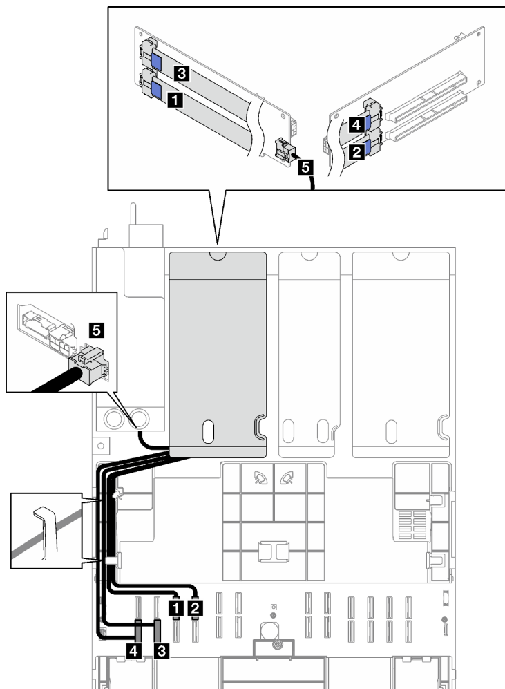
Figure 167. Cheminement des câbles pour la carte mezzanine PCIe 3 à deux emplacements
