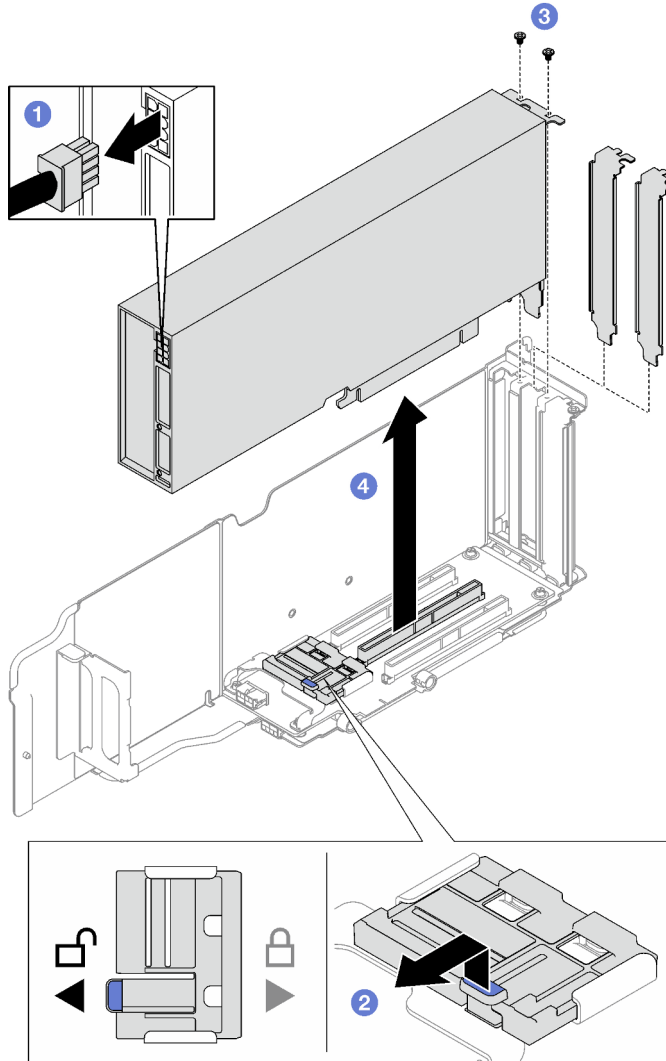
Figure 48. Retrait d'un adaptateur GPU double largeur
