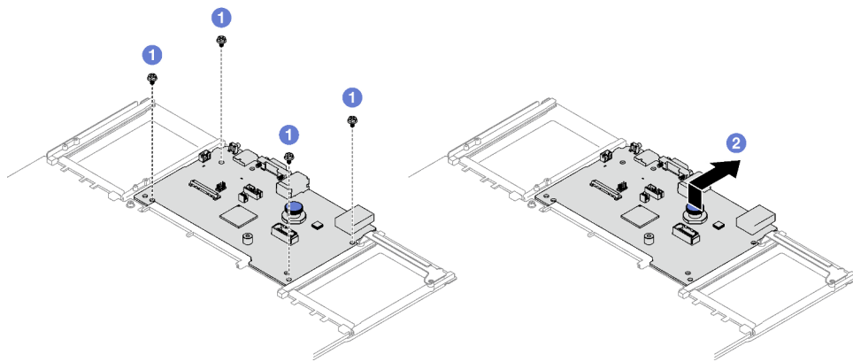
Figure 133. Retrait de la carte d'E-S système
