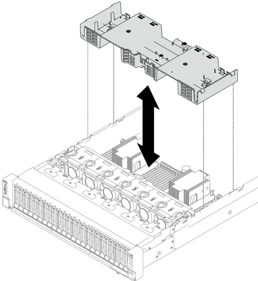
Figure 18. Installation de la grille d'aération avant
