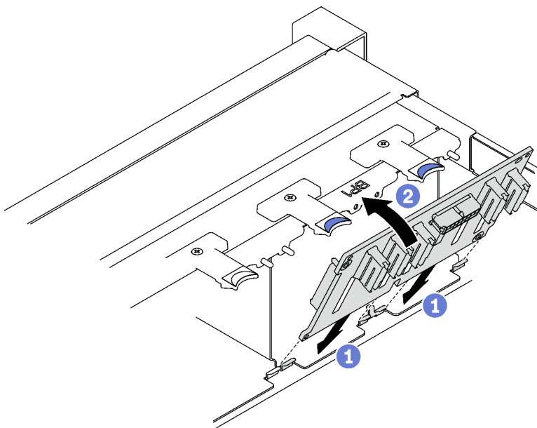
Figure 6. Installation d'un fond de panier d'unité 2,5 pouces
