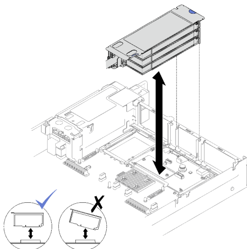
Figure 81. Installation d'une carte mezzanine PCIe LP (sans connecteur d'alimentation)
