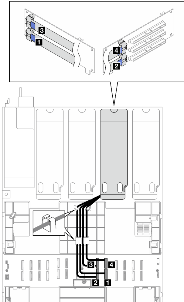
Figure 170. Cheminement des câbles pour la carte mezzanine PCIe B
