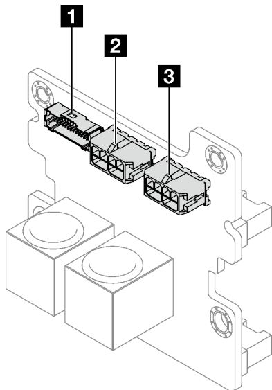
Figure 149. Connecteurs du tableau de distribution
