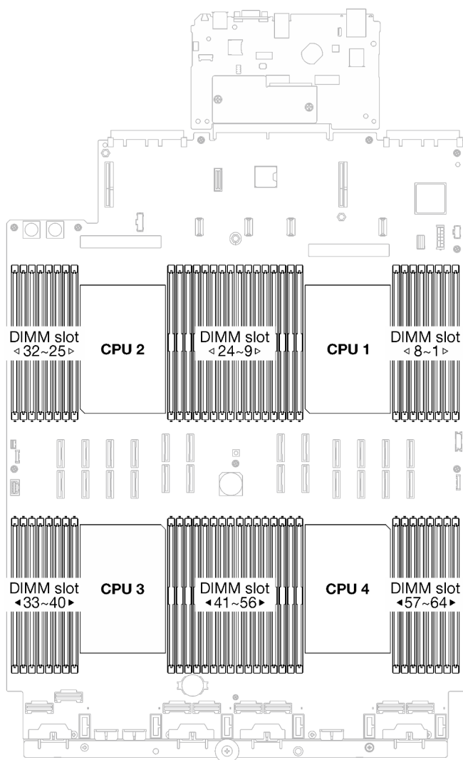
Figure 67. Disposition des modules de mémoire et des processeurs
