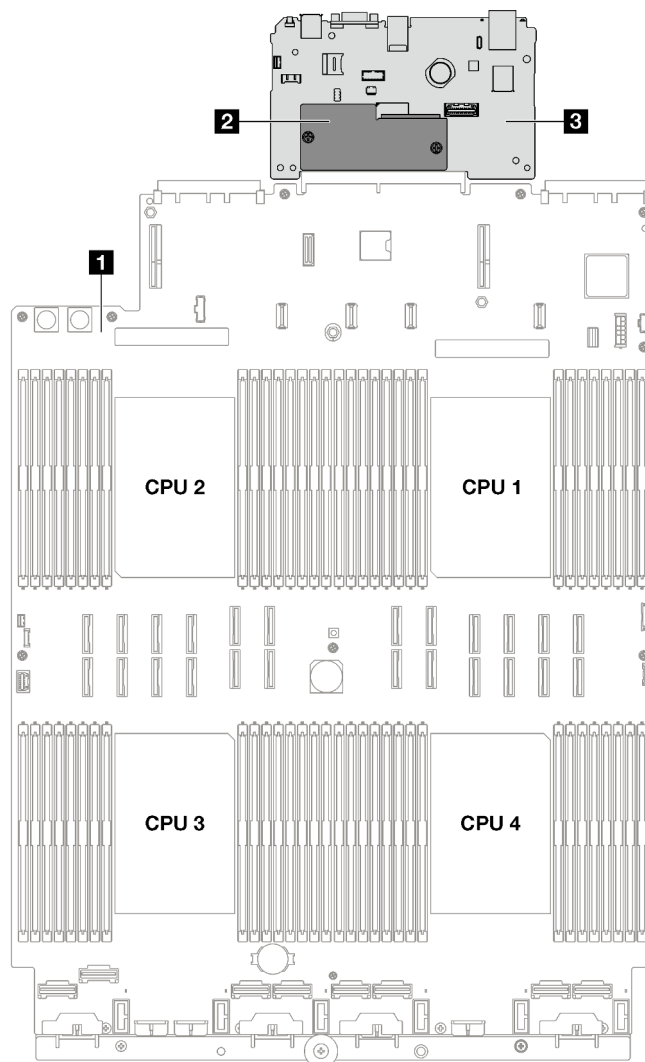
Figure 129. Disposition du bloc carte mère
