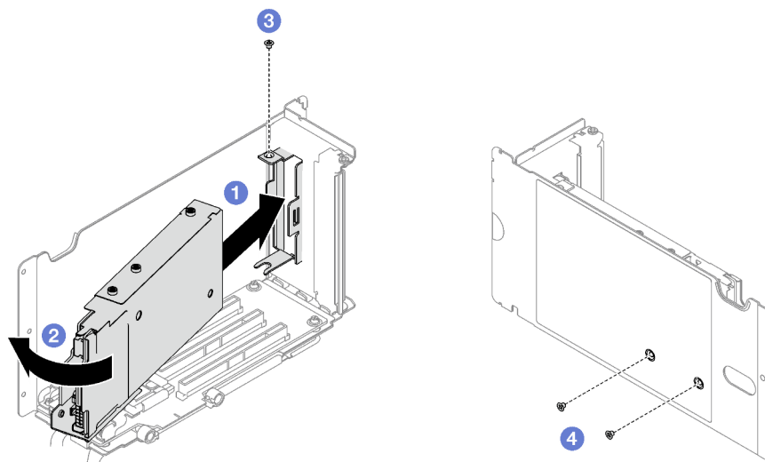
Figure 12. Installation du boîtier d'unités de disque dur 7 mm
