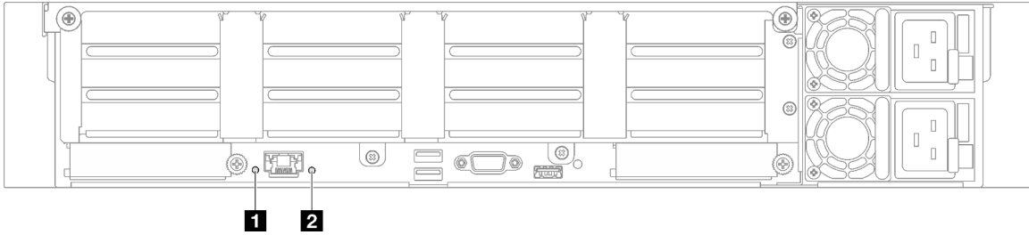
Figure 182. Voyants système au niveau de la vue arrière - Modèle de serveur doté de quatre cartes mezzanines PCIe
