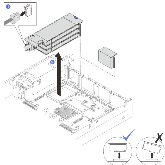
Figure 74. Retrait d'une carte mezzanine PCIe LP (avec connecteur d'alimentation)
