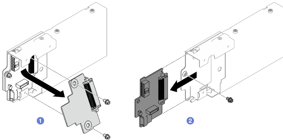
Figure 10. Retrait du fond de panier d'unité 7 mm
