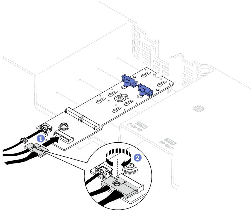
Figure 27. Connexion des câbles de fond de panier M.2 SATA/NVMe
