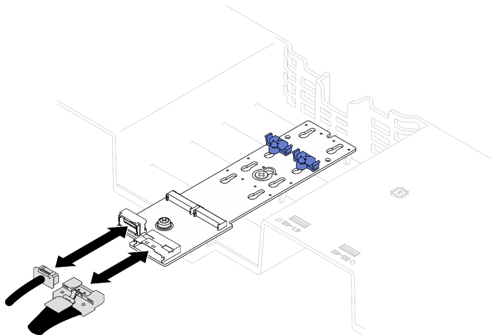
Figure 24. Déconnexion des câbles du fond de panier M.2 SATA/x4 NVMe
