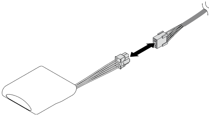
Figure 46. Connexion du câble du module d'alimentation flash
