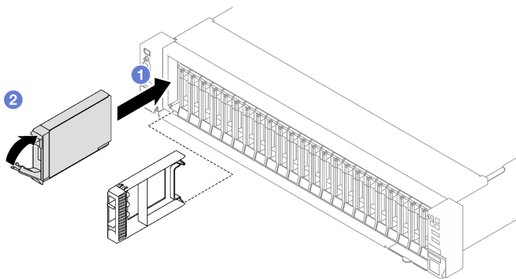
Figure 7. Installation d'une unité remplaçable à chaud 2,5 pouces
