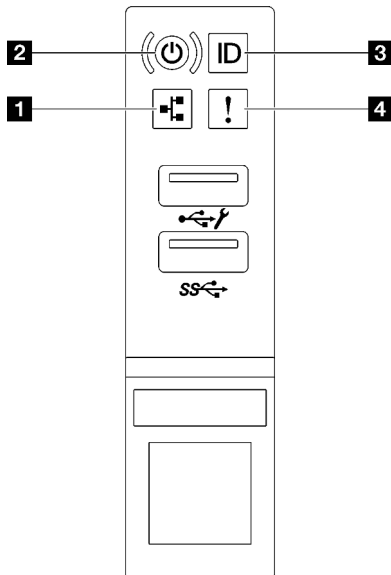
Figure 178. Voyants du module d'E-S avant
