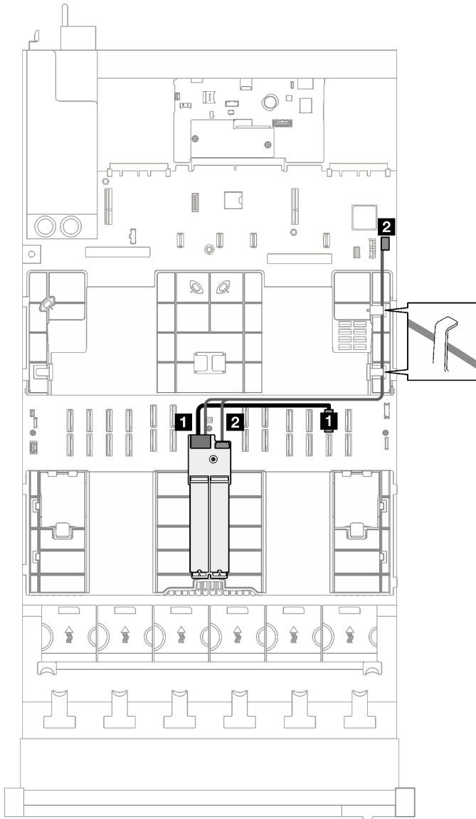
Figure 157. Cheminement des câbles pour le fond de panier M.2 SATA/x4 NVMe vers le processeur
