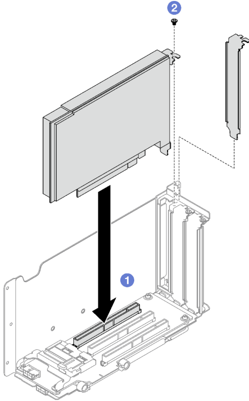
Figure 78. Installer un adaptateur PCIe
