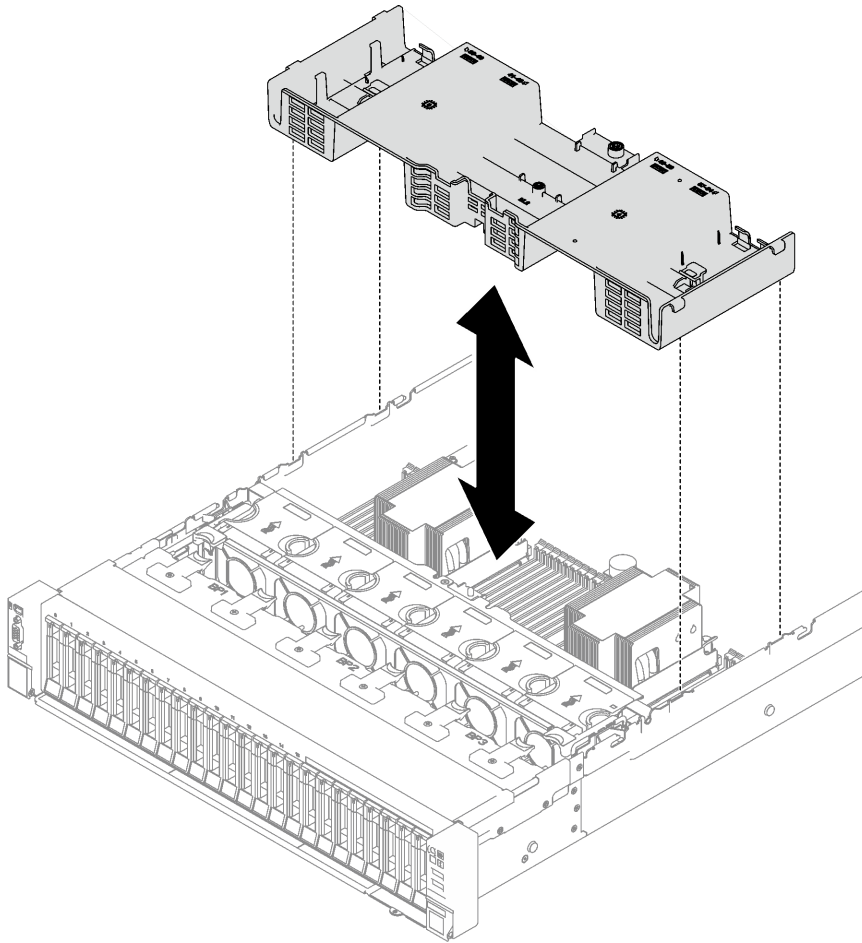
Figure 17. Retrait de la grille d'aération avant
