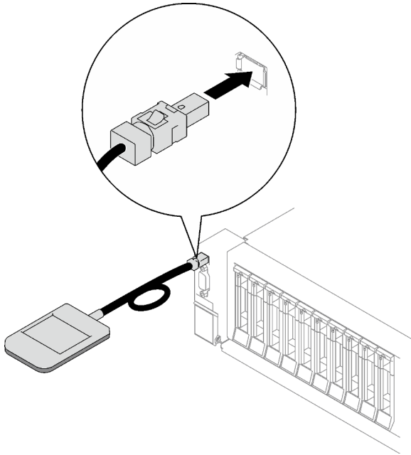
Figure 36. Connexion du câble de l'ensemble de diagnostics externe
