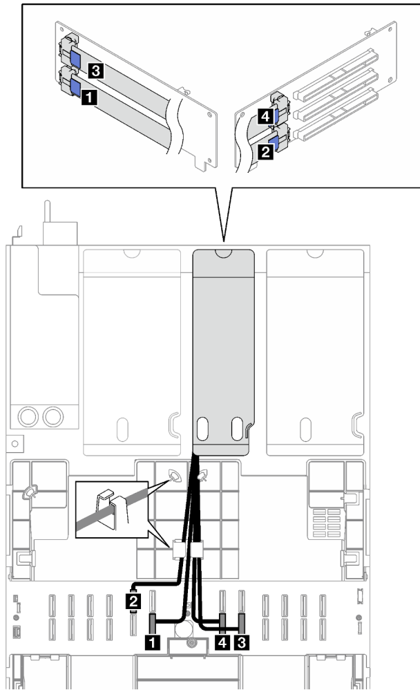
Figure 165. Cheminement des câbles pour le bloc mezzanine PCIe 2 à trois emplacements
