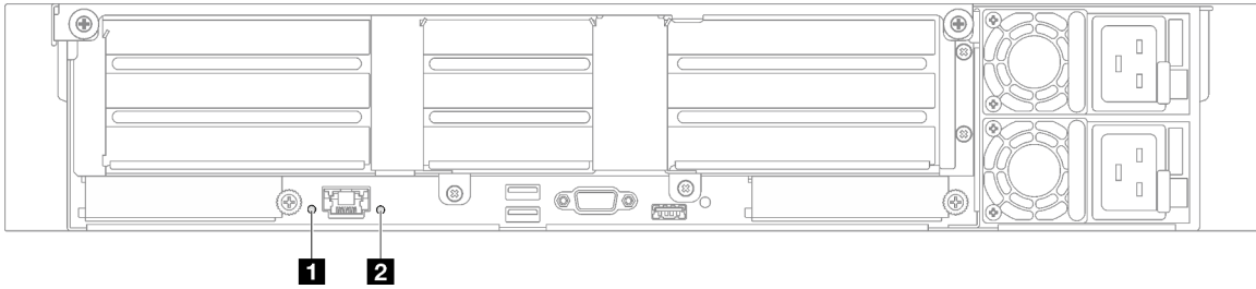
Figure 181. Voyants système au niveau de la vue arrière - Modèle de serveur doté de trois cartes mezzanines PCIe
