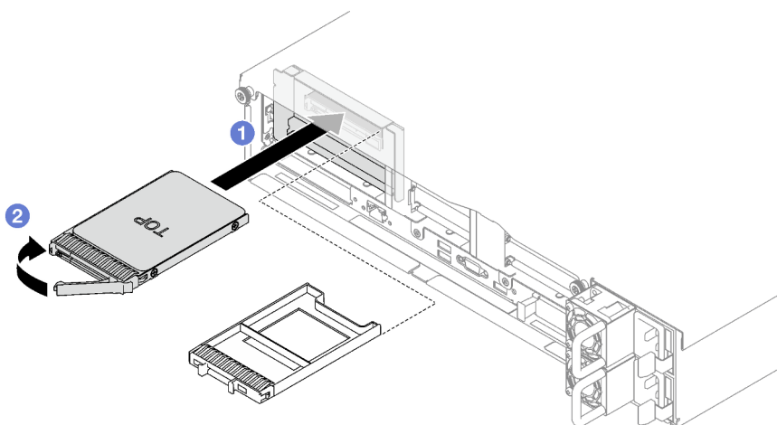
Figure 13. Installation de l'unité 7 mm
