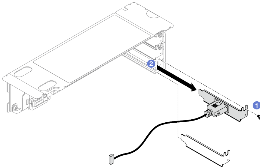
Figure 126. Retrait du module de port série
