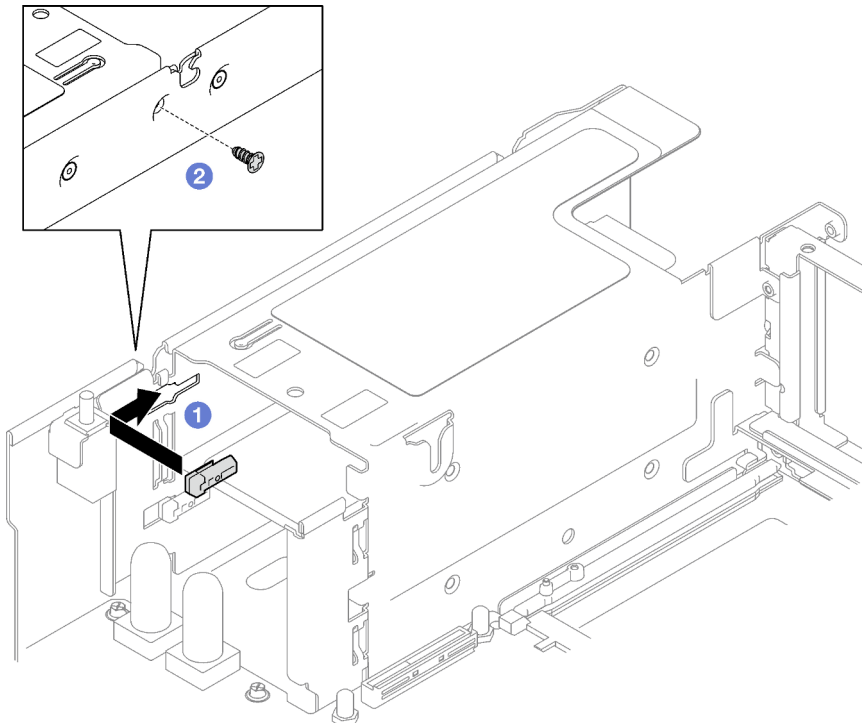
Figure 108. Installation de la clé d'alimentation
