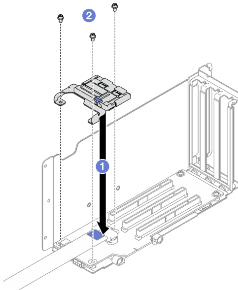
Figure 97. Installation du dispositif de retenue PCIe
