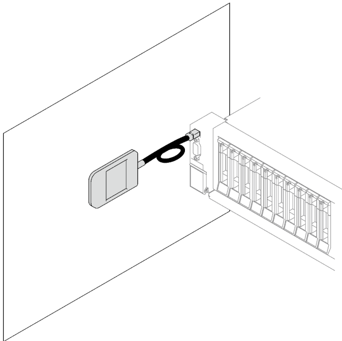
Figure 37. Fixation de l'ensemble de diagnostics externe à une surface métallique
