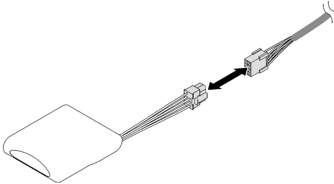
Figure 14. Déconnexion du câble du module d'alimentation flash
