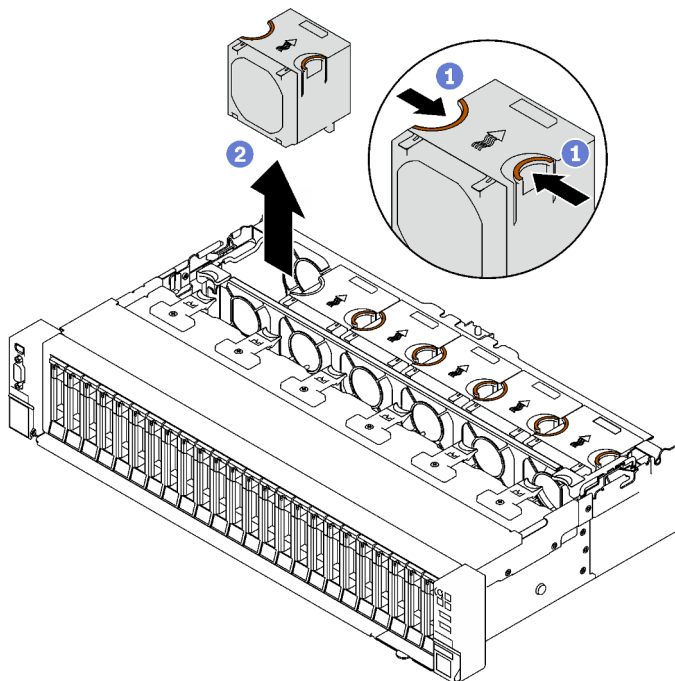
Figure 38. Retrait du ventilateur
