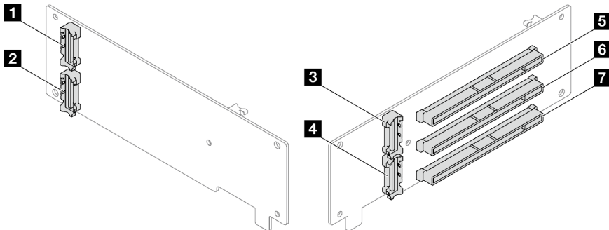
Figure 147. Connecteurs de carte mezzanine PCIe Gen4 à trois emplacements (sans connecteur d'alimentation)
