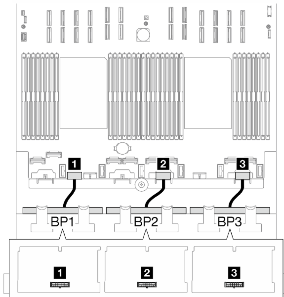
Figure 152. Cheminement des câbles d'alimentation pour les fonds de panier d'unité 2,5 pouces
