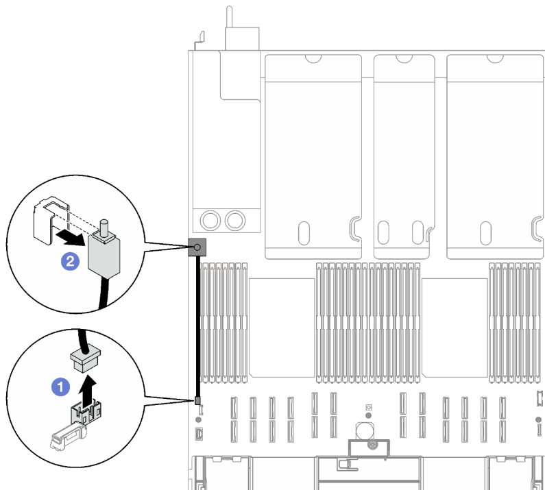
Figure 51. Retrait du commutateur de détection d'intrusion
