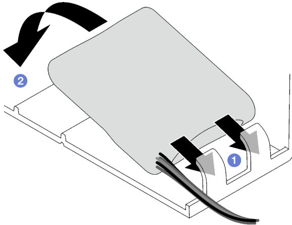
Figure 45. Installation du module d'alimentation flash
