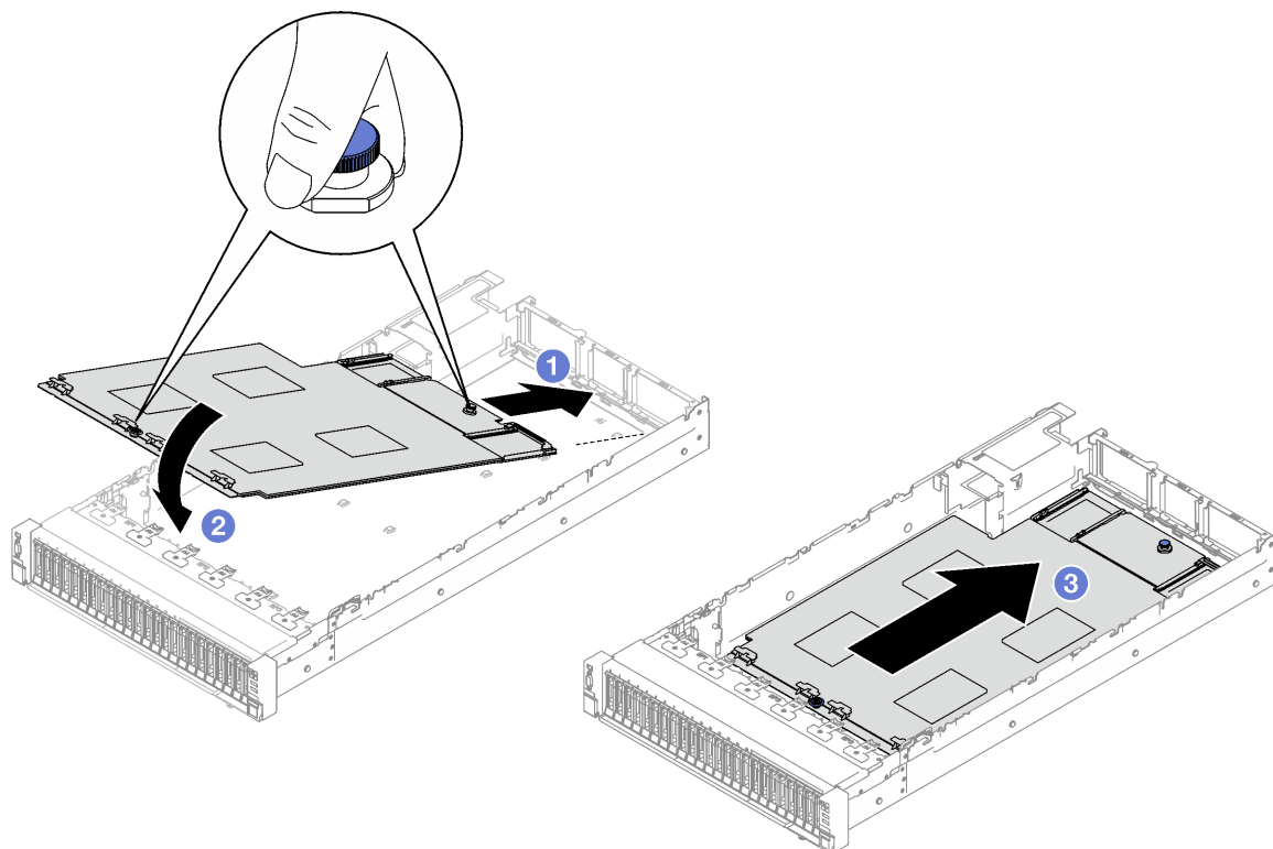
Figure 135. Installation du bloc carte mère
