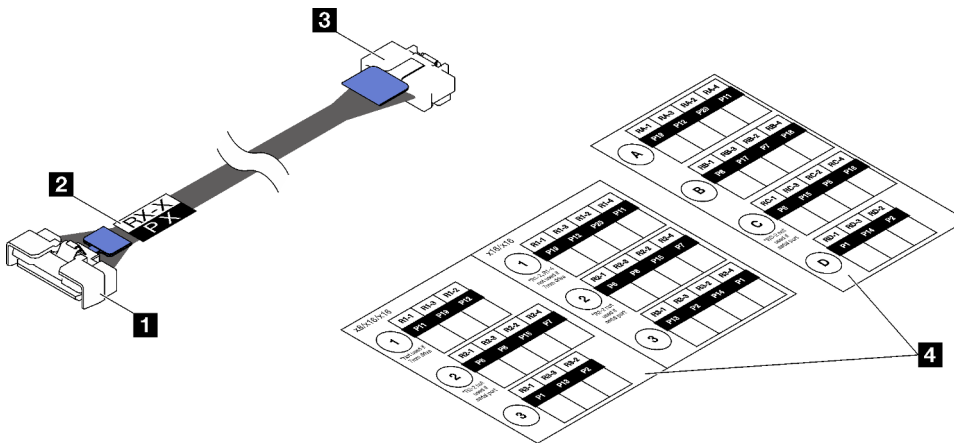
Figure 89. Cordon d'alimentation de carte mezzanine PCIe
