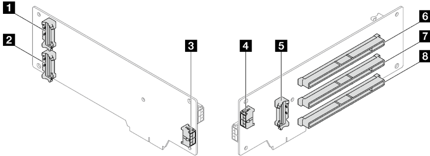
Figure 146. Connecteurs de carte mezzanine PCIe Gen5 à trois emplacements (avec connecteur d'alimentation)
