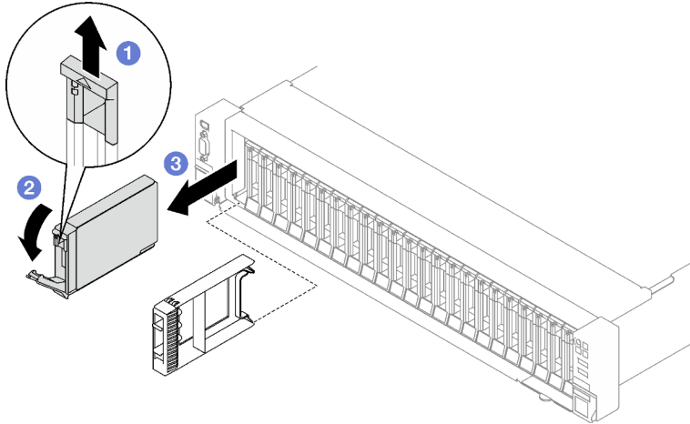
Figure 3. Retrait d'une unité remplaçable à chaud 2,5 pouces
