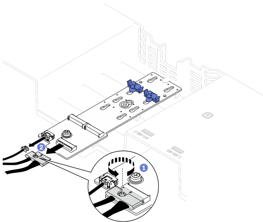
Figure 55. Déconnexion du câble du fond de panier SATA/NVMe ou NVMe M.2
