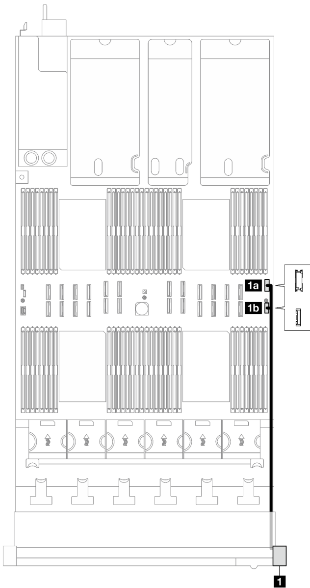
Figure 154. Cheminement des câbles du module d'E-S avant
