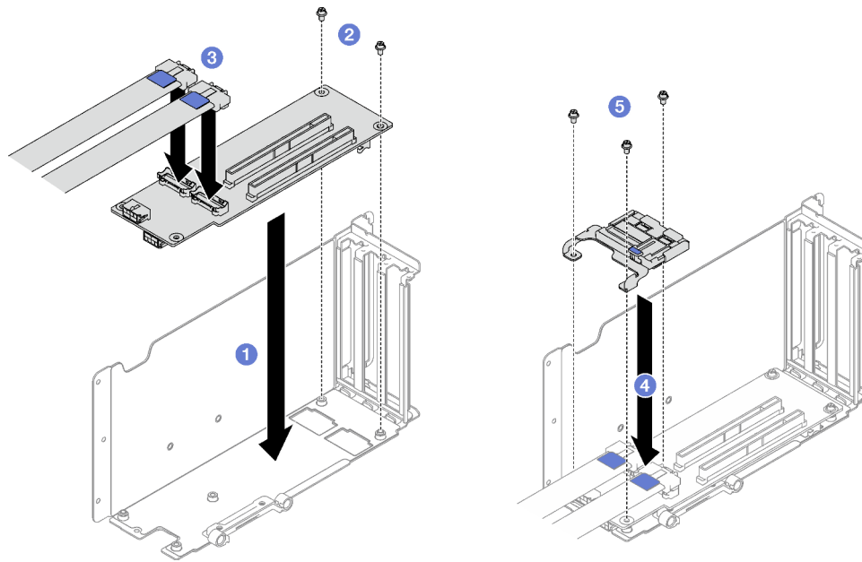
Figure 92. Installation d'une carte mezzanine PCIe
