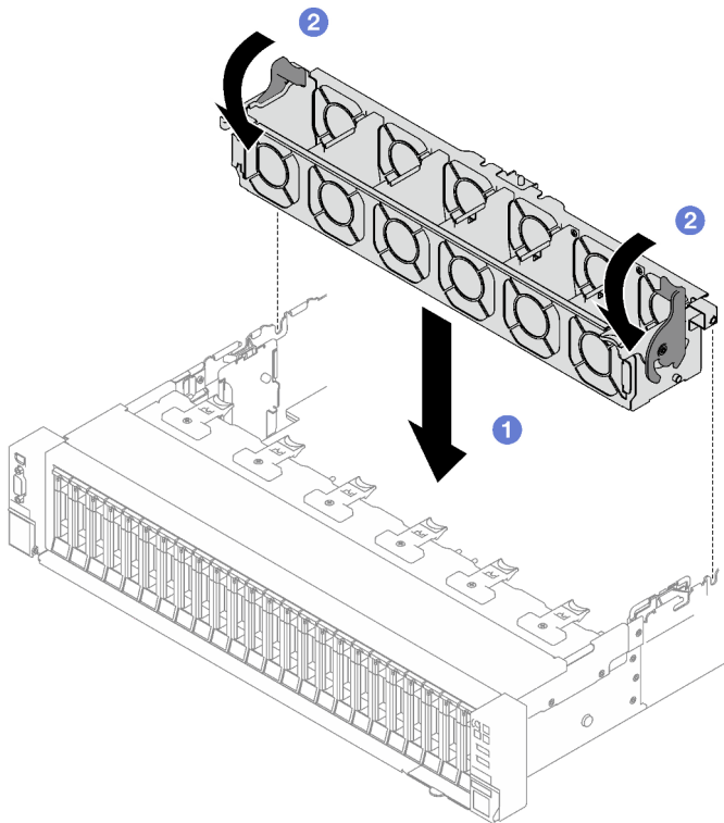
Figure 40. Installation du boîtier de ventilation
