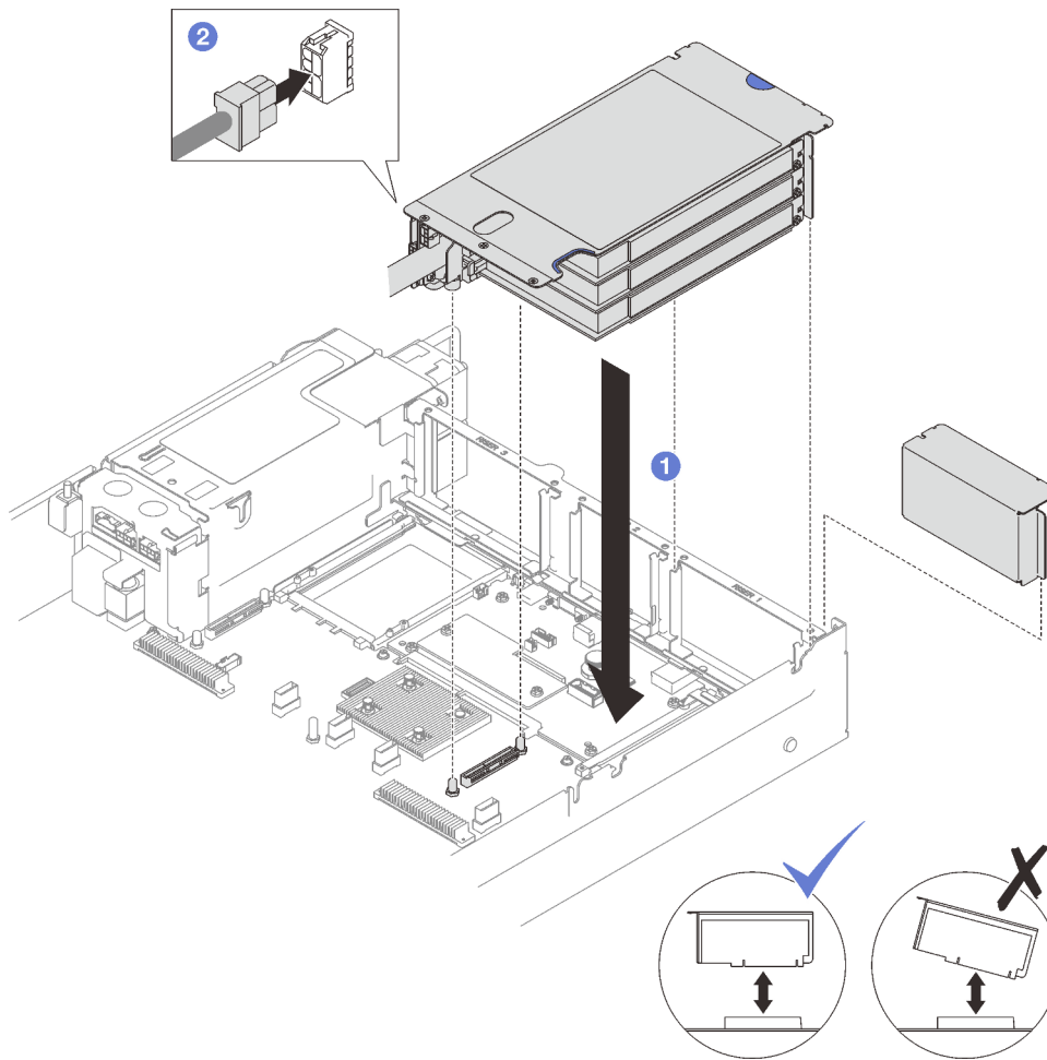
Figure 83. Installation d'une carte mezzanine PCIe FHHL
