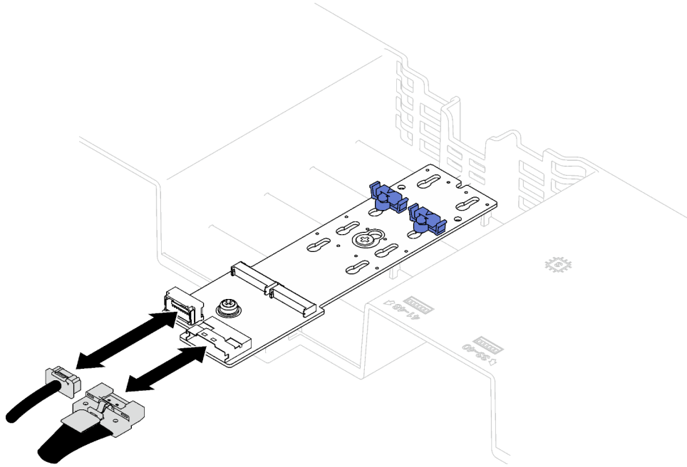
Figure 58. Connexion des câbles de fond de panier M.2 SATA/x4 NVMe
