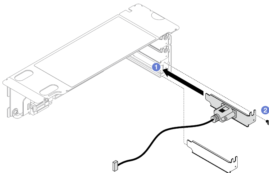
Figure 127. Installation du module de port série
