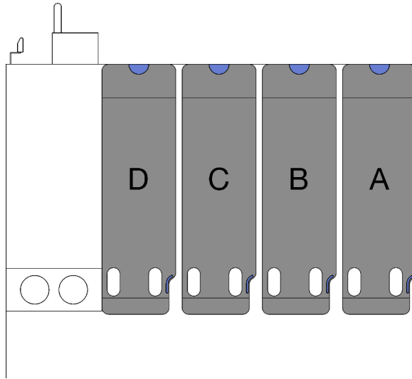
Figure 80. Type et emplacement de carte mezzanine PCIe pour le modèle de serveur doté de quatre cartes mezzanines PCIe
