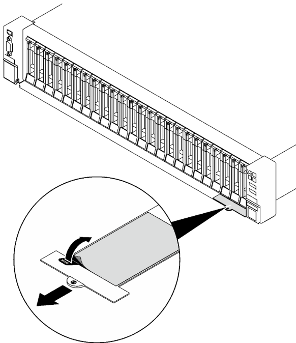
Figura 29. Etichetta di accesso alla rete di Lenovo XClarity Controller sulla scheda informativa estraibile
