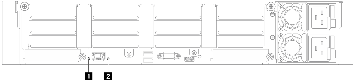
Figura 24. LED di sistema sulla vista posteriore - Modello di server con quattro schede verticali PCIe
