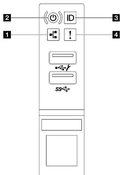
Figura 20. LED del modulo I/O anteriore
