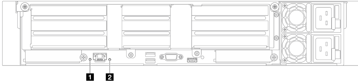
Figura 23. LED di sistema sulla vista posteriore - Modello di server con tre schede verticali PCIe
