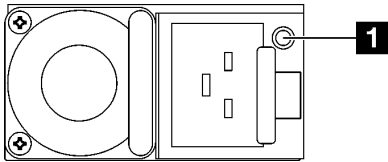
Figura 22. LED dell'alimentatore CRPS
