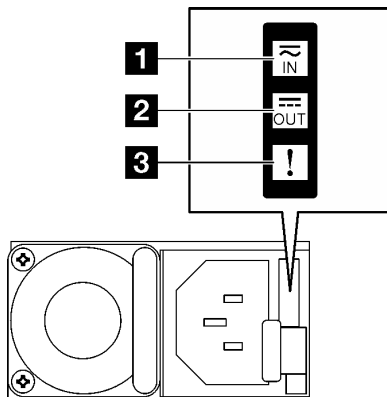
Figura 21. LED dell'alimentatore CFFv4
