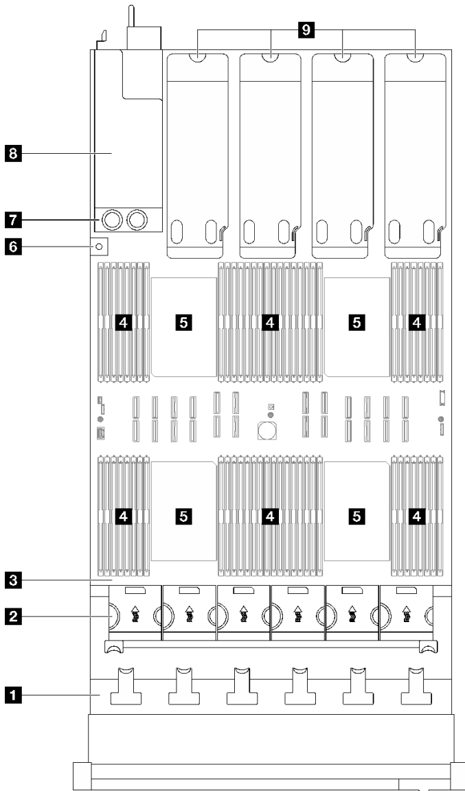
그림 14. PCIe 라이저 4개가 지원되는 서버 모델의 평면도
