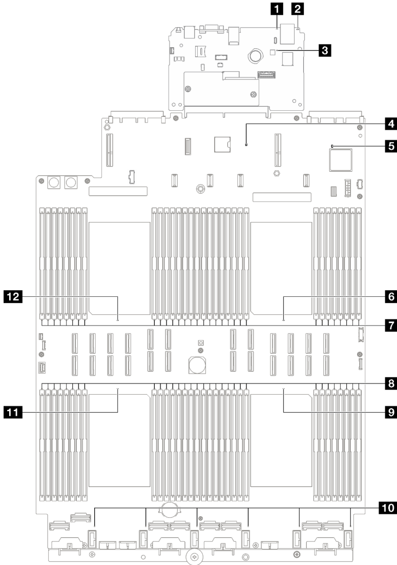
그림 25. 시스템 보드 어셈블리 LED
