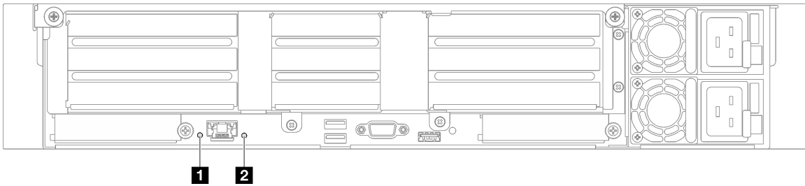
그림 23. 뒷면의 시스템 LED - PCIe 라이저 3개가 지원되는 서버 모델
