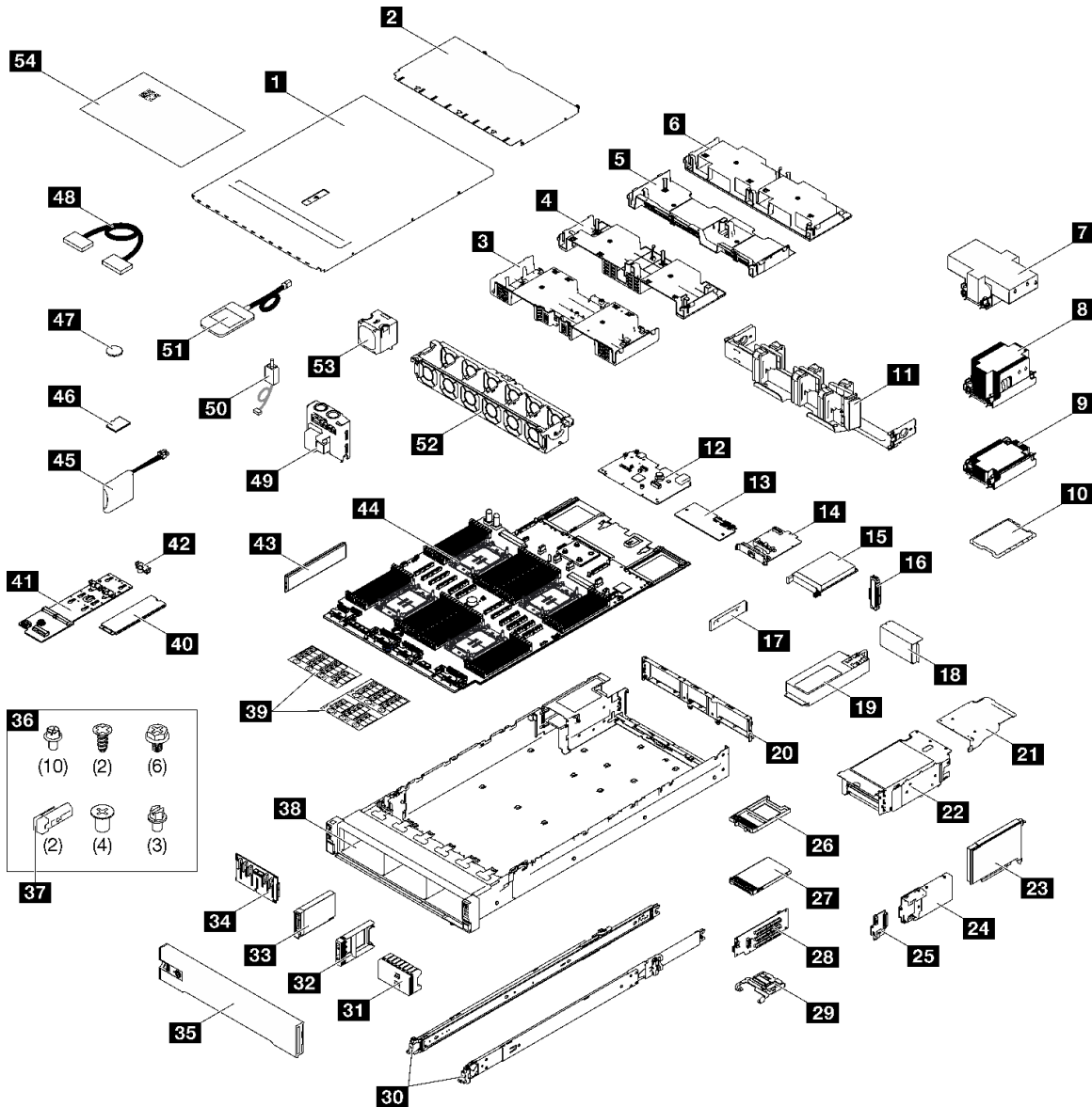
그림 27. 서버 구성 요소
