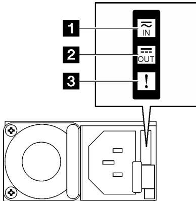
그림 21. CFFv4 전원 공급 장치 LED
