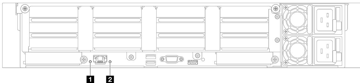
图 24. 后视图上的系统 LED - 配备四个 PCIe 转接卡的服务器型号
