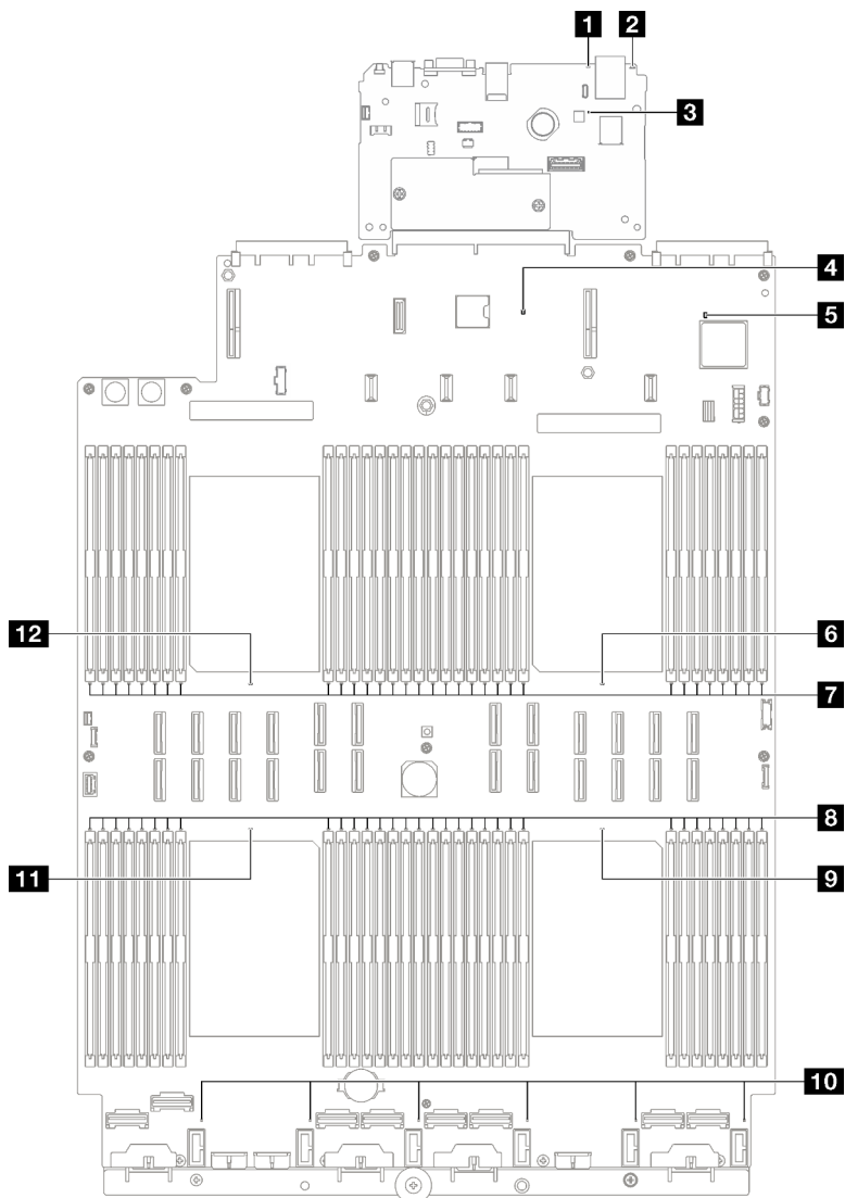
图 25. 主板组合件 LED
