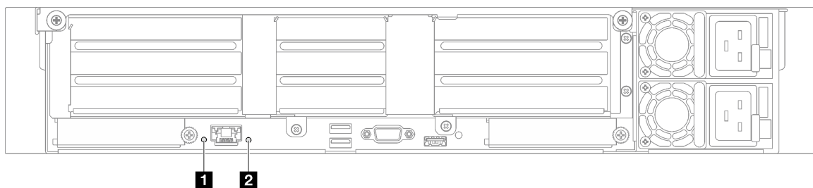
图 23. 后视图上的系统 LED - 配备三个 PCIe 转接卡的服务器型号
