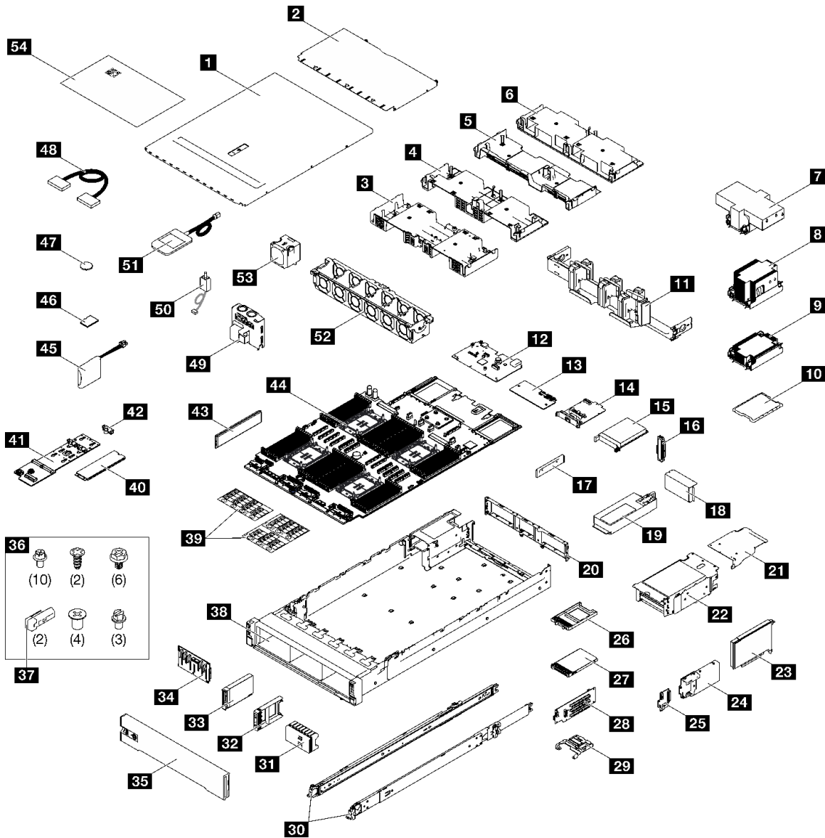
图 27. 服务器组件
