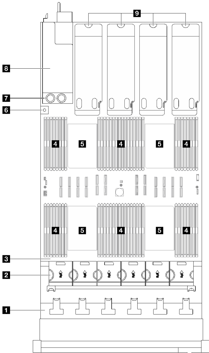
圖例 14. 配備四個 PCIe 擴充卡之伺服器型號的俯視圖
