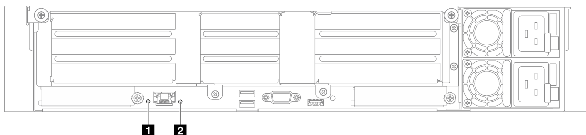
圖例 23. 背面圖上的系統 LED - 配備三個 PCIe 擴充卡的伺服器型號
