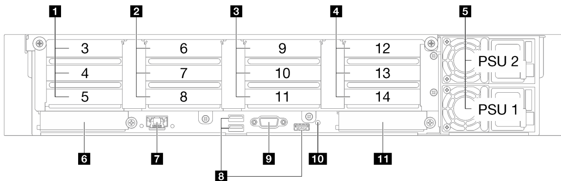
圖例 8. 配備四個 PCIe 擴充卡之伺服器型號的背面圖
