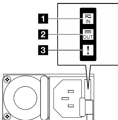
圖例 21. CFFv4 電源供應器 LED
