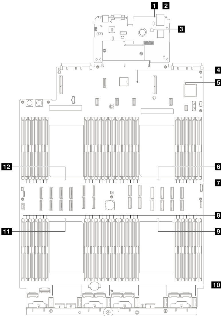
圖例 25. 主機板組件 LED
