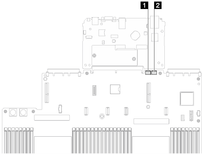
圖例 18. 主機板組件開關
