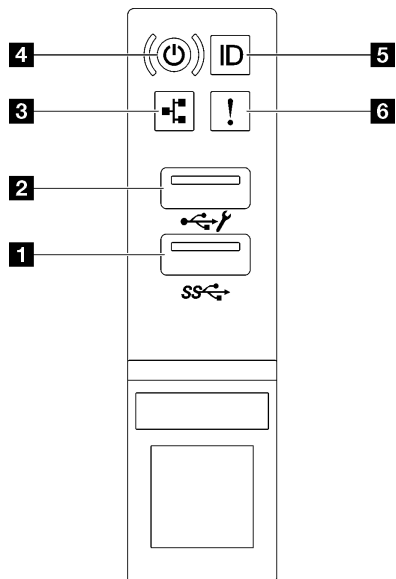
圖例 15. 正面 I/O 模組
