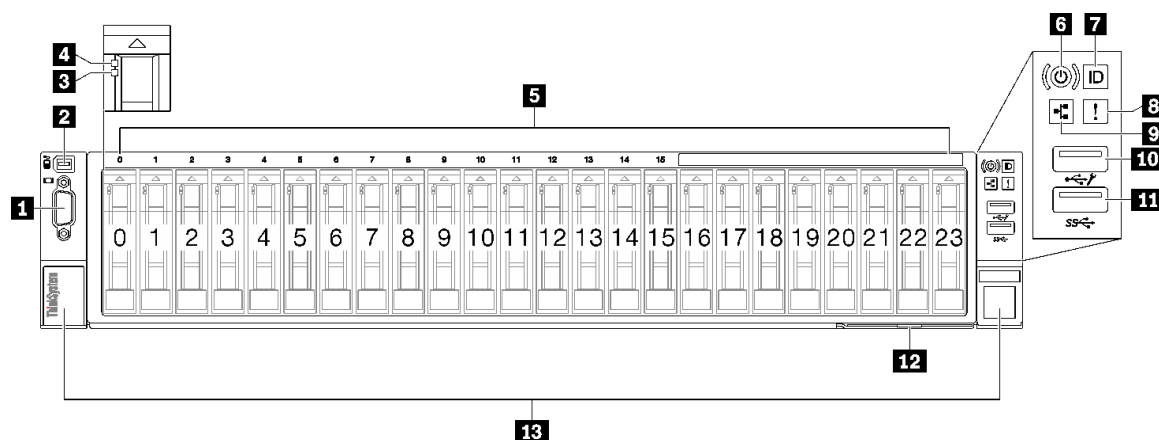
圖例 2. 配備 2.5 吋硬碟之伺服器型號的正面圖
