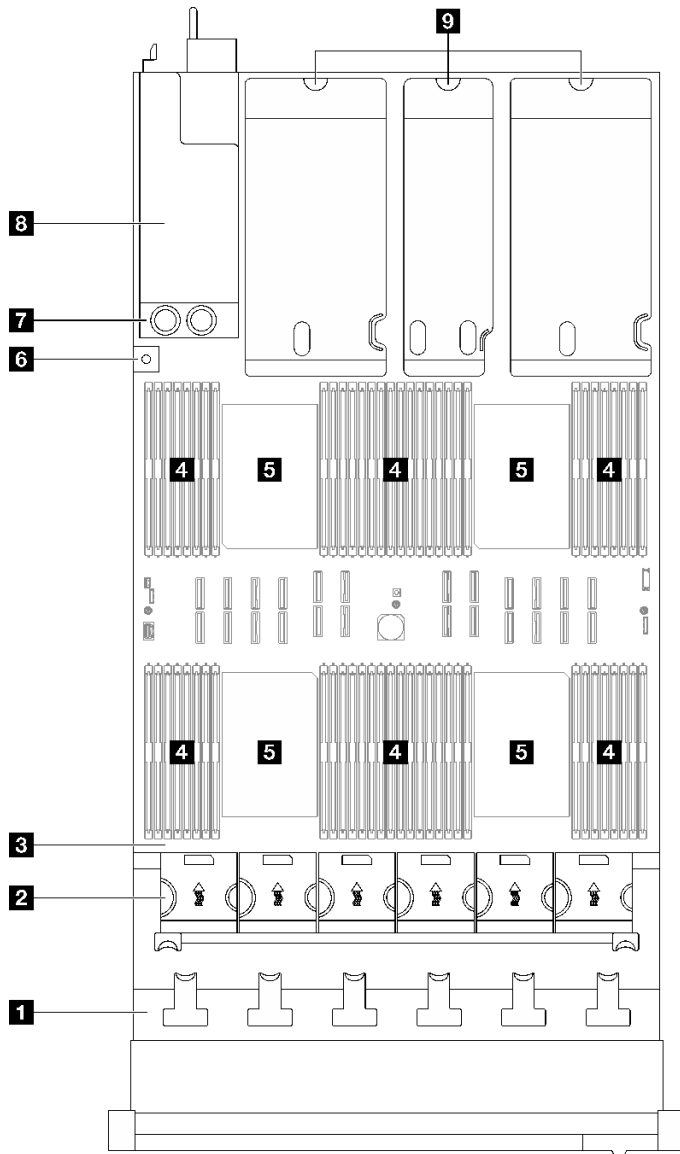
圖例 13. 配備三個 PCIe 擴充卡之伺服器型號的俯視圖
