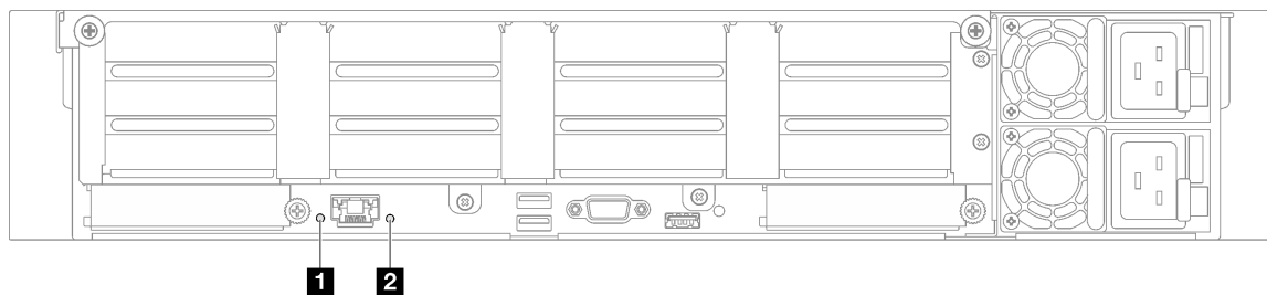
圖例 24. 背面圖上的系統 LED - 配備四個 PCIe 擴充卡的伺服器型號
