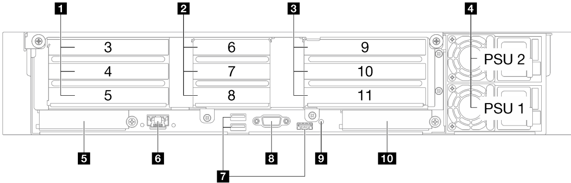
圖例 3. 配備三個 PCIe 擴充卡之伺服器型號的背面圖
