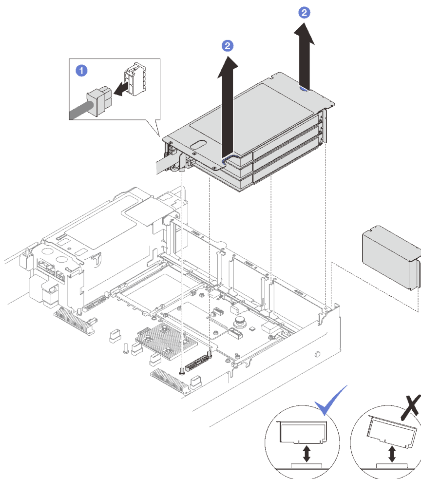
圖例 97. 卸下 PCIe FHHL 擴充卡
