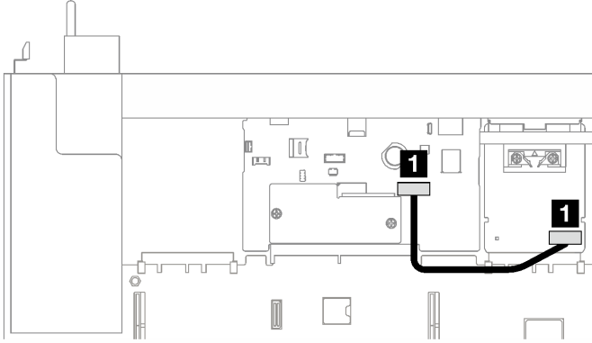
圖例 180. 管理 NIC 配接卡的纜線佈線
