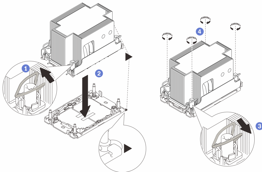
圖例 140. 2U 標準 PHM 安裝
