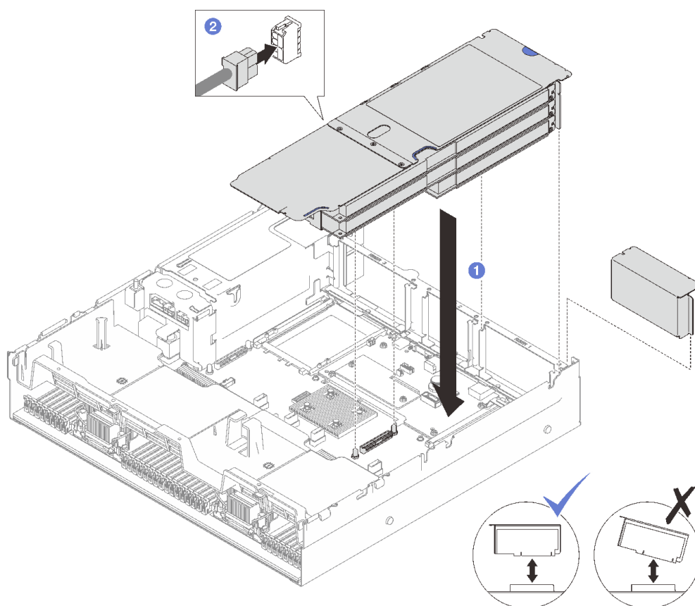
圖例 106. 安裝 PCIe FHFL 擴充卡
