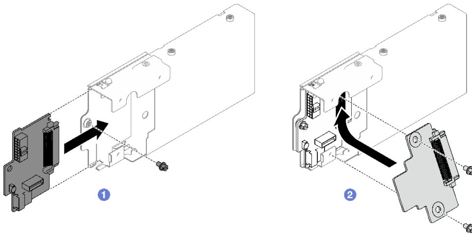
圖例 33. 安裝 7 公釐硬碟背板
