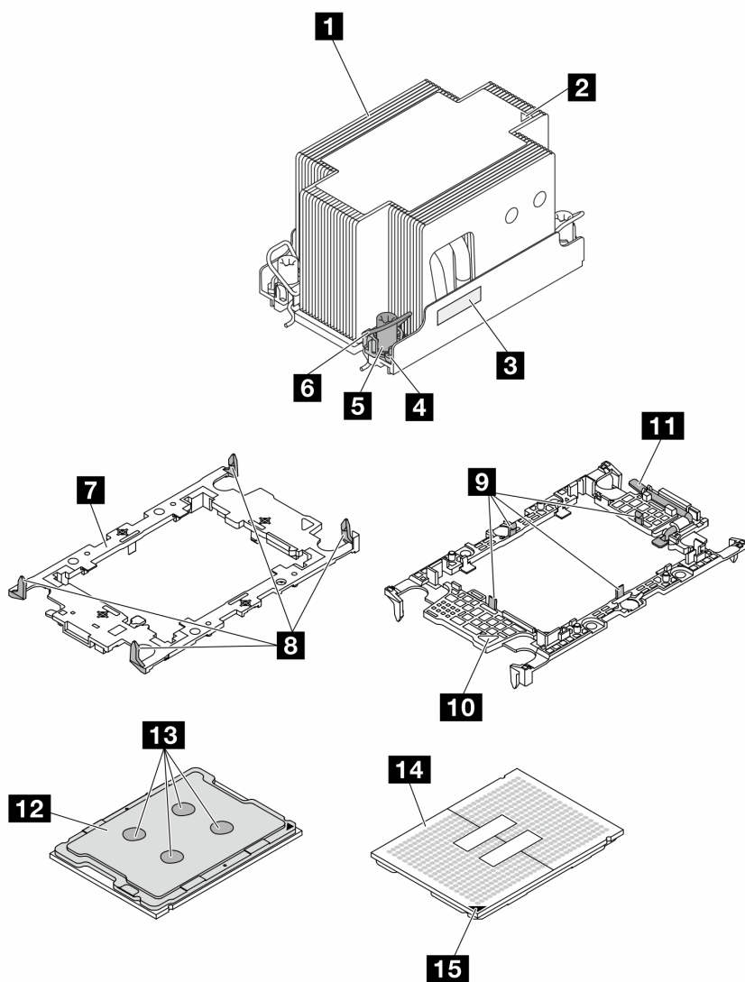
圖例 131. PHM 元件
