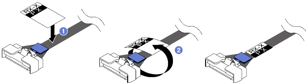
圖例 112. 黏貼標籤
