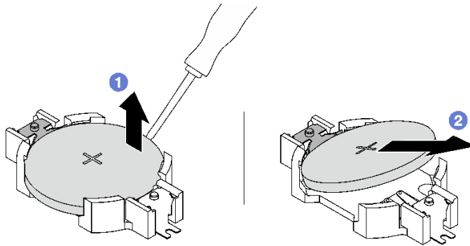
圖例 54. 卸下 CMOS 電池
