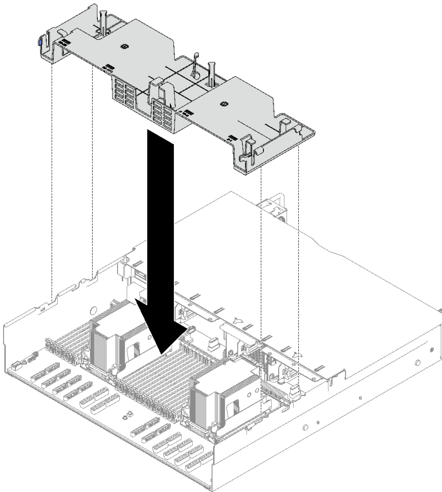
圖例 48. 安裝後方空氣擋板
