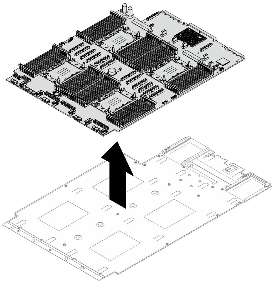
圖例 210. 拆卸處理器板
