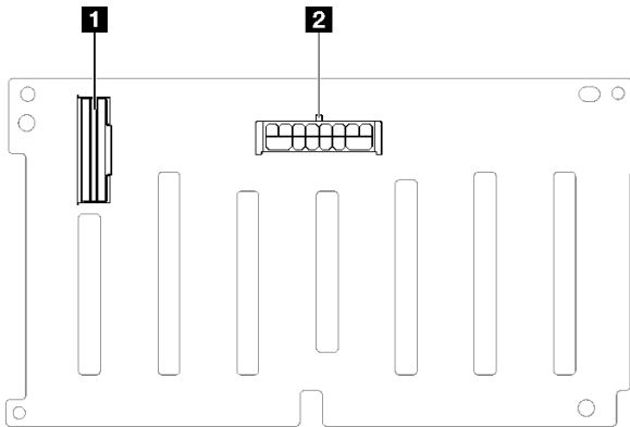
圖例 164. 8x 2.5 吋 SAS/SATA 背板接頭
