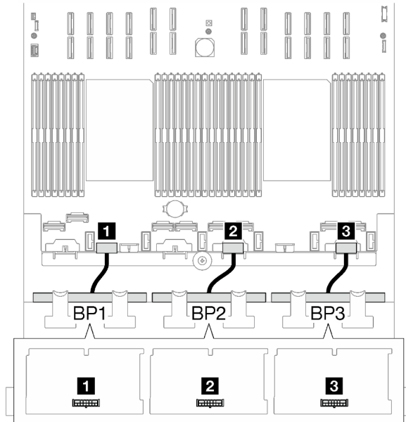
圖例 174. 2.5 吋硬碟背板的電源線纜線佈線
