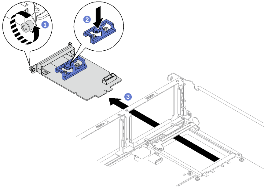
圖例 85. 卸下管理 NIC 配接卡
