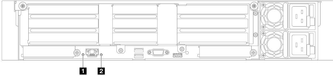
圖例 202. 背面圖上的系統 LED - 配備三個 PCIe 擴充卡的伺服器型號
