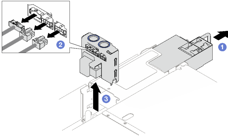
圖例 122. 卸下電源配送板
