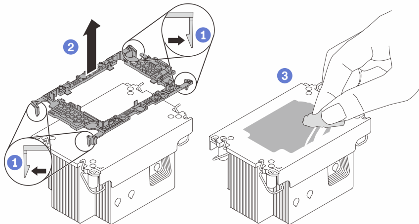
圖例 135. 將處理器支架與散熱槽分開
