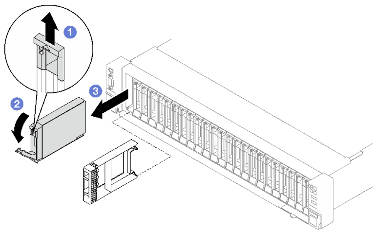
圖例 25. 卸下 2.5 吋熱抽換硬碟
