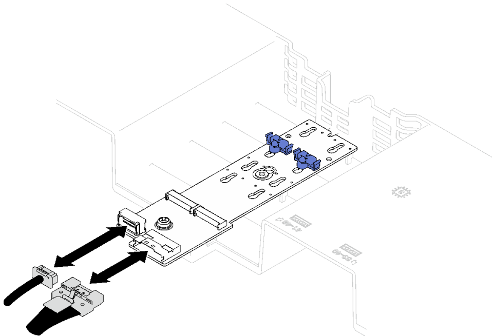
圖例 50. 連接 SATA/x4 NVMe M.2 背板纜線
