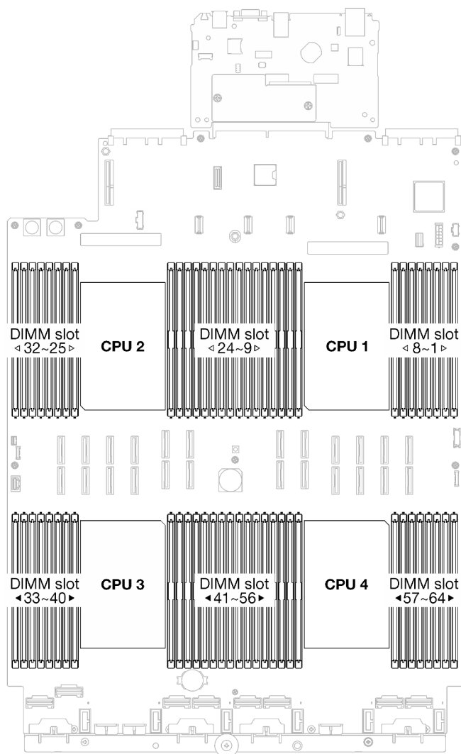
圖例 89. 記憶體模組和處理器佈置
