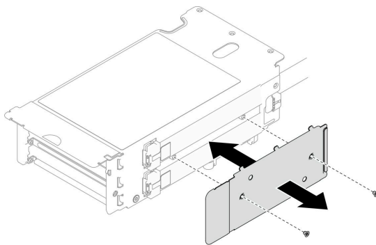
圖例 107. 卸下纜線蓋
