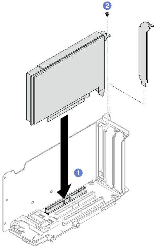
圖例 100. PCIe 配接卡安裝
