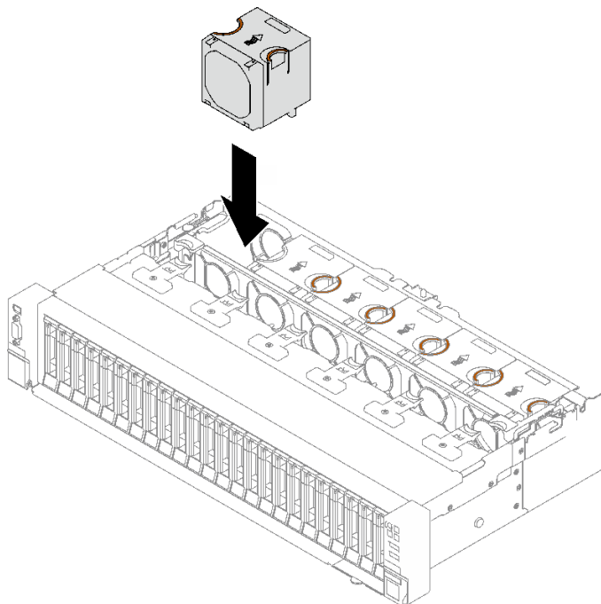
圖例 63. 安裝風扇
