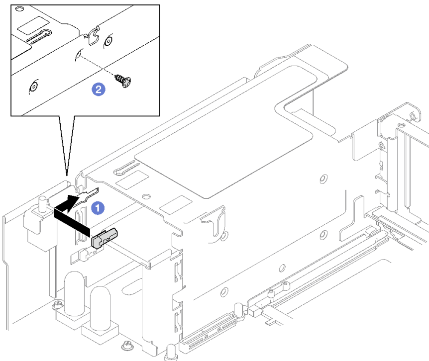
圖例 130. 安裝電源供應器鑰匙
