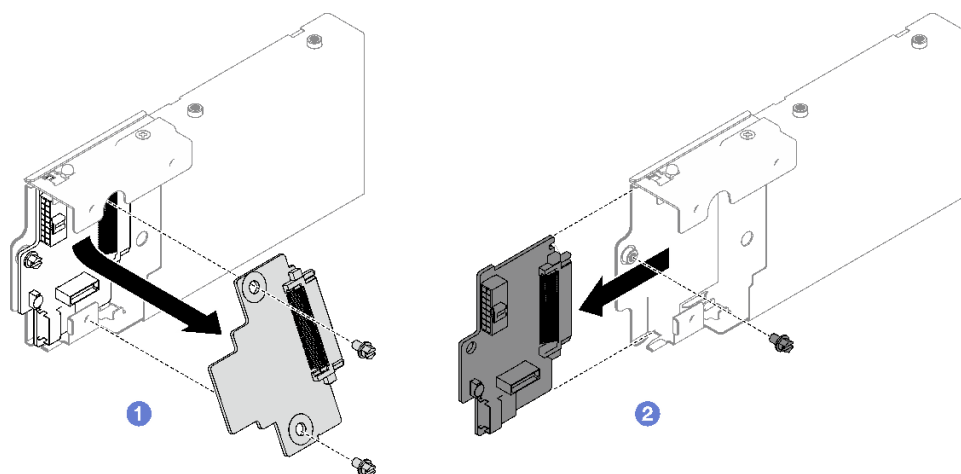
圖例 32. 卸下 7 公釐硬碟背板
