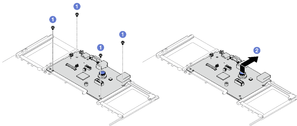
圖例 207. 卸下系統 I/O 板
