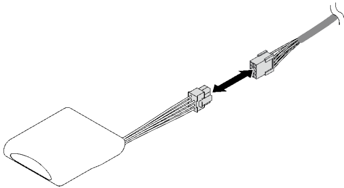
圖例 64. 拔掉快閃記憶體電源模組纜線
