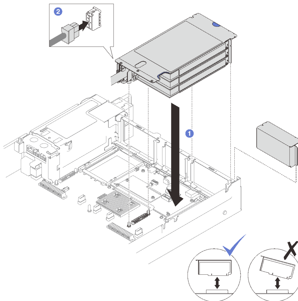
圖例 105. 安裝 PCIe FHHL 擴充卡
