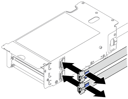
圖例 115. 纜線連接
