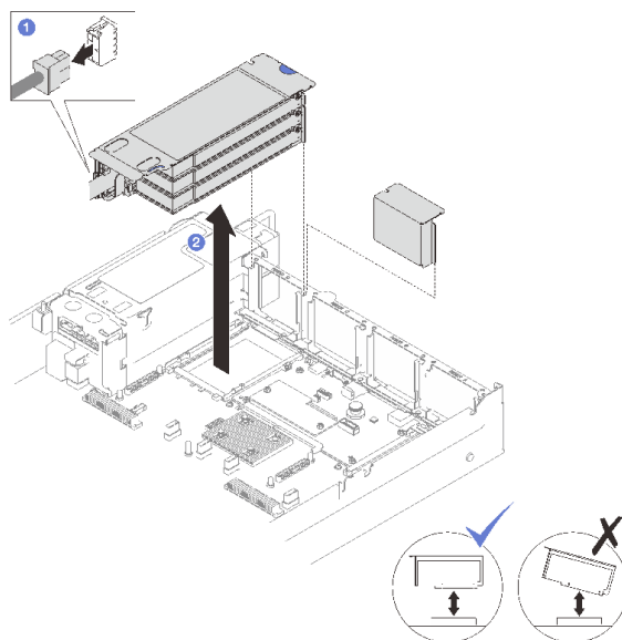
圖例 96. 卸下 PCIe LP 擴充卡 (含電源線)
