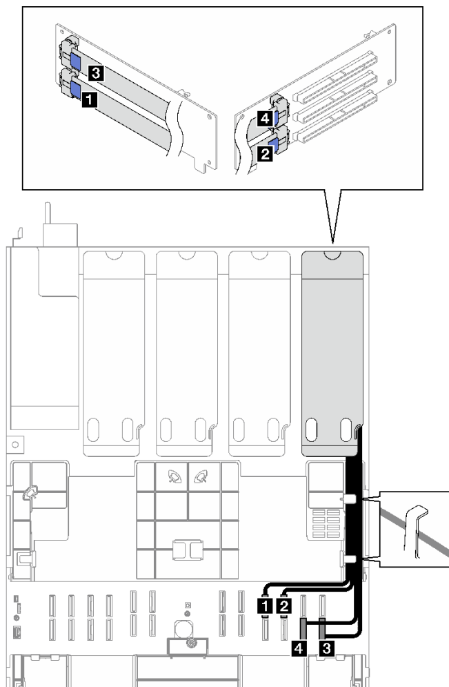
圖例 191. PCIe 擴充卡 A 的纜線佈線
