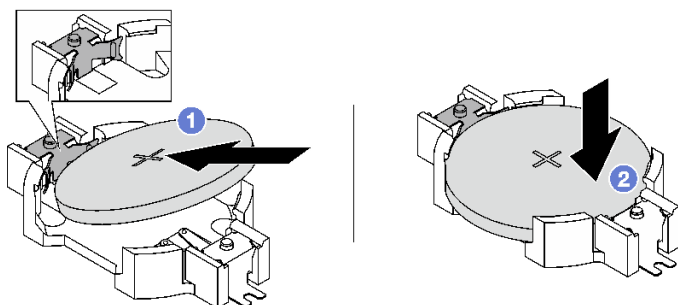
圖例 56. CMOS 電池安裝
