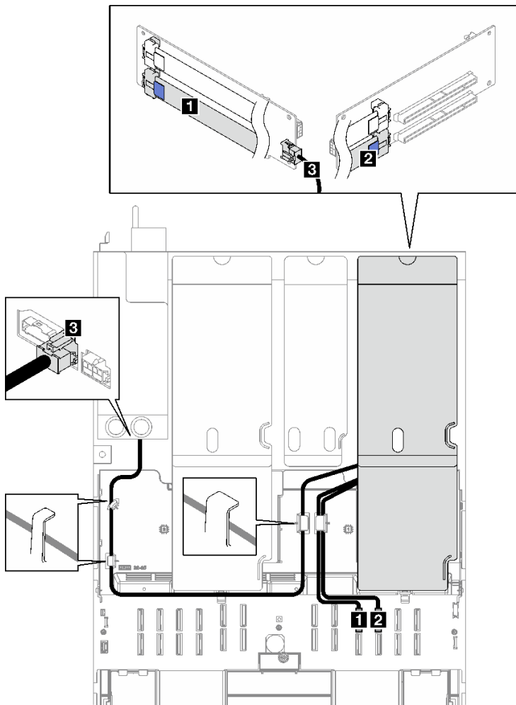
圖例 184. 雙插槽 PCIe FL 擴充卡 1 ( 含 7 公釐框架 ) 的纜線佈線
