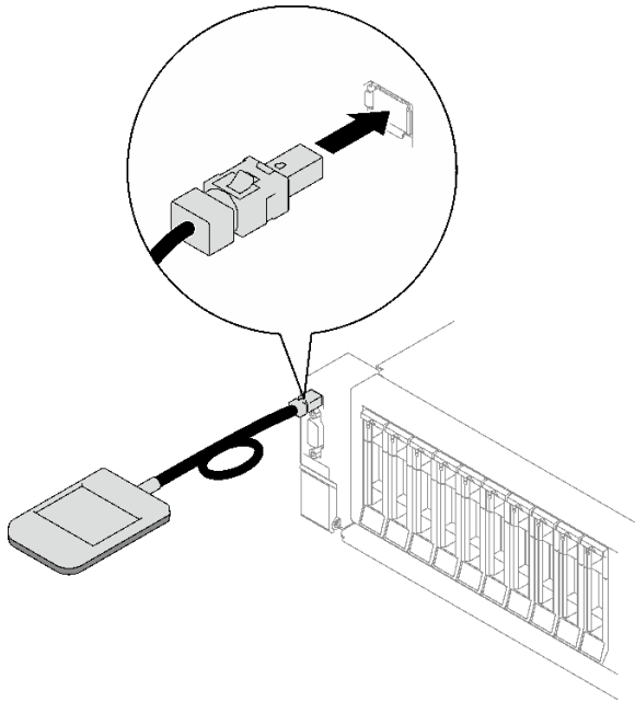
圖例 58. 連接外部診斷手持裝置纜線
