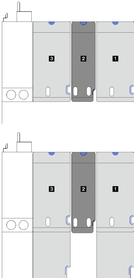
圖例 101. 配備三個 PCIe 擴充卡之伺服器型號的 PCIe 擴充卡類型和位置
