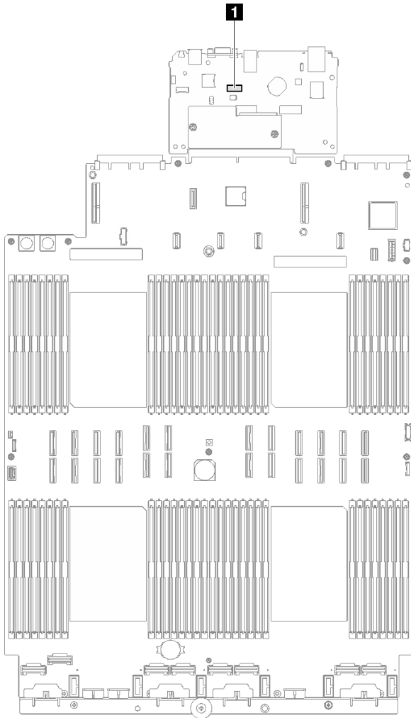
圖例 150. 序列埠接頭位置
