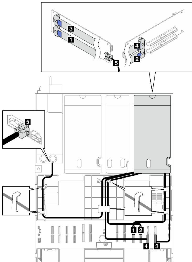
圖例 181. 雙插槽 PCIe HL 擴充卡 1 的纜線佈線
