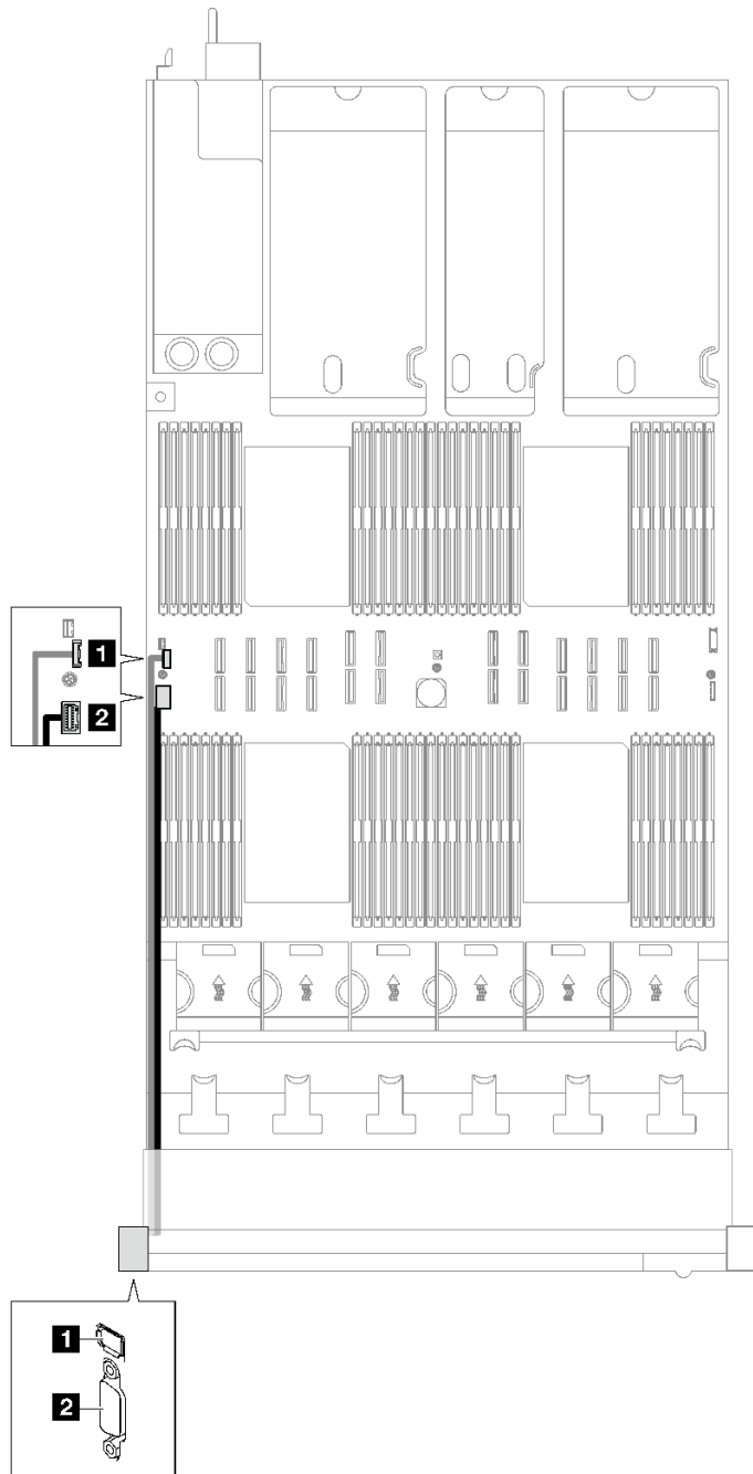
圖例 175. 外部診斷手持裝置和 VGA 的纜線佈線
