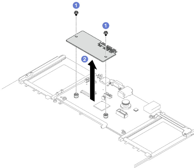
圖例 152. 卸下韌體和 RoT 安全模組
