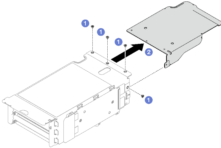
圖例 120. 卸下 PCIe 擴充卡延伸器
