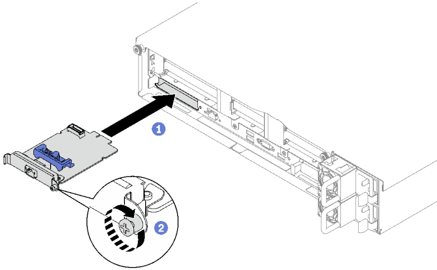
圖例 86. 安裝管理 NIC 配接卡
