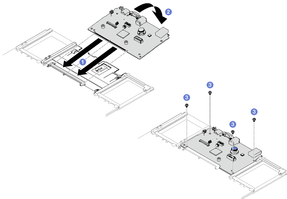
圖例 156. 安裝系統 I/O 板
