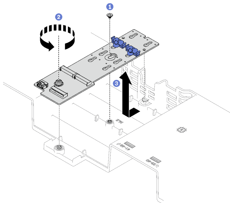
圖例 76. 卸下 M.2 背板
