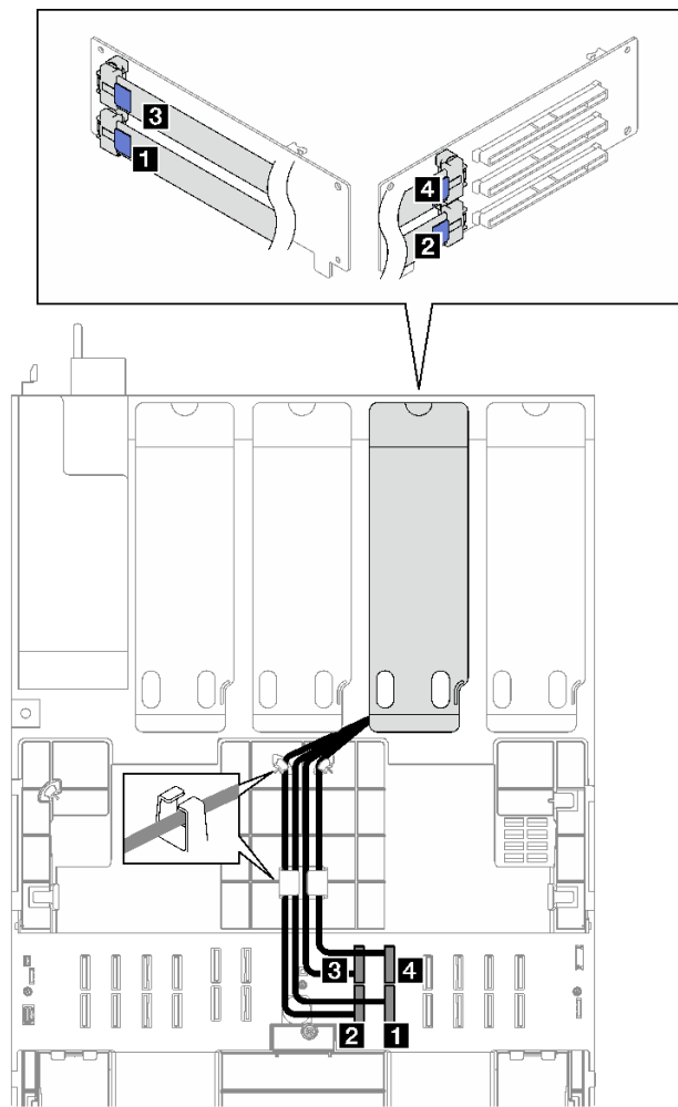
圖例 192. PCIe 擴充卡 B 的纜線佈線
