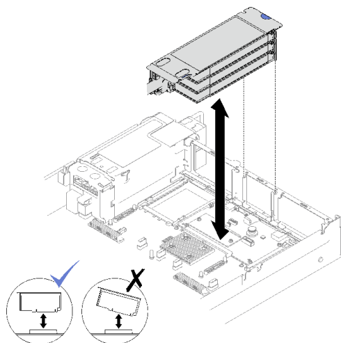
圖例 95. 卸下 PCIe LP 擴充卡 (不含電源線)
