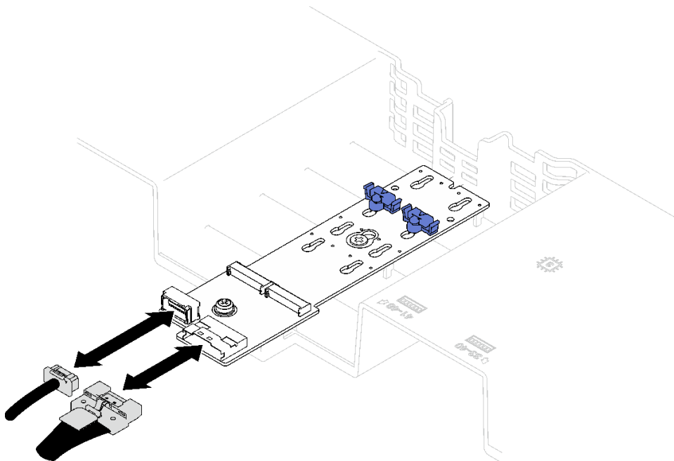
圖例 38. 拔除 SATA/x4 NVMe M.2 背板纜線
