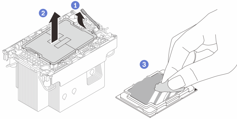
圖例 134. 將處理器與散熱槽和支架分開
