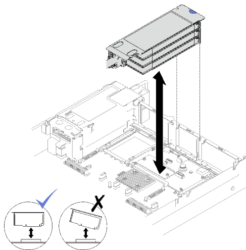
圖例 103. 安裝 PCIe LP 擴充卡（不含電源線）
