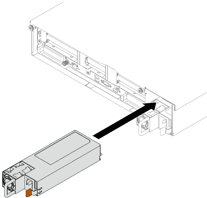
圖例 126. 安裝電源供應器
