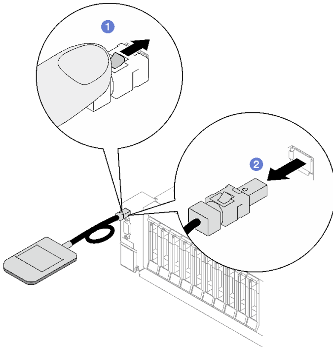
圖例 57. 拔掉外部診斷手持裝置纜線
