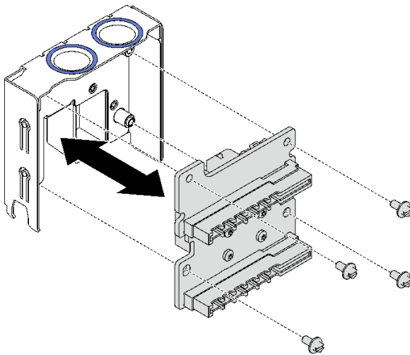
圖例 123. 拆卸電源配送板
