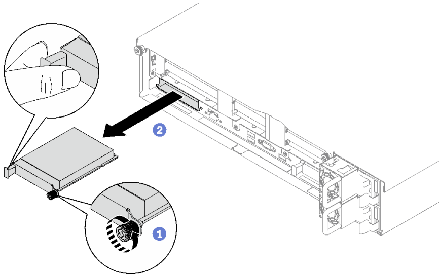
圖例 93. 卸下 OCP 模組
