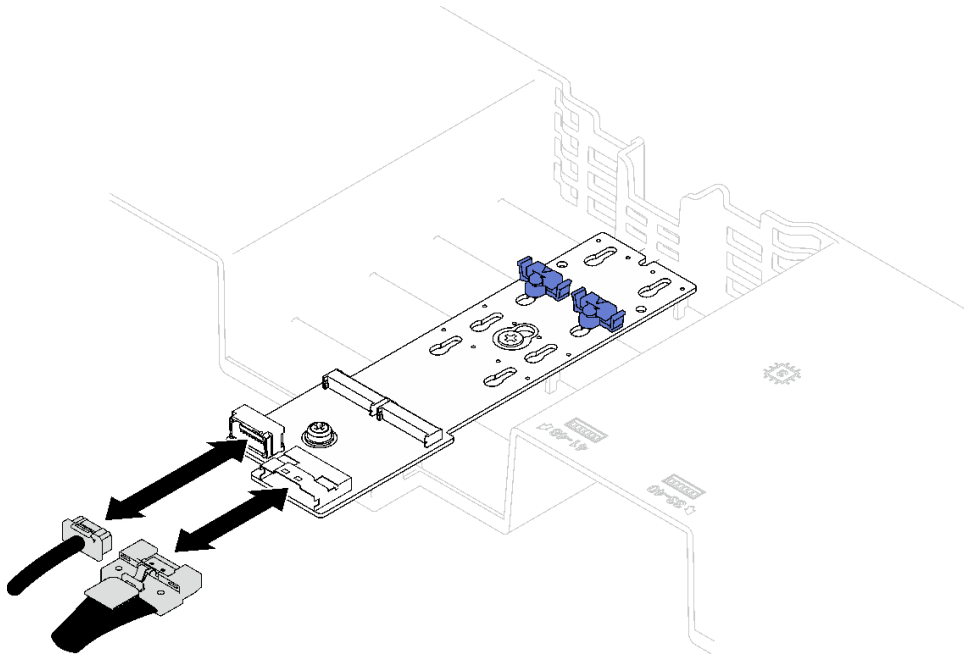
圖例 80. 連接 SATA/x4 NVMe M.2 背板纜線
