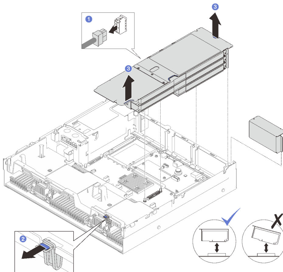
圖例 98. 卸下 PCIe FHFL 擴充卡
