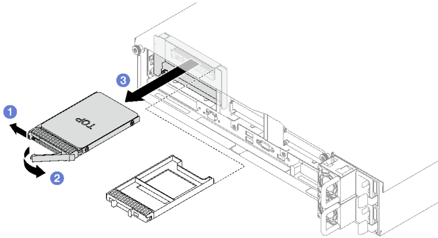
圖例 30. 卸下 7 公釐硬碟
