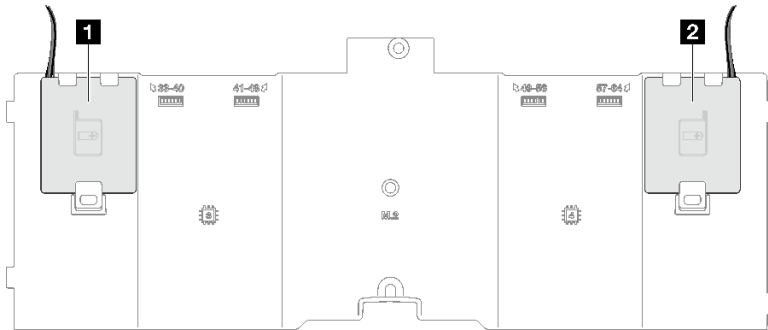
圖例 66. 快閃記憶體電源模組插槽位置
