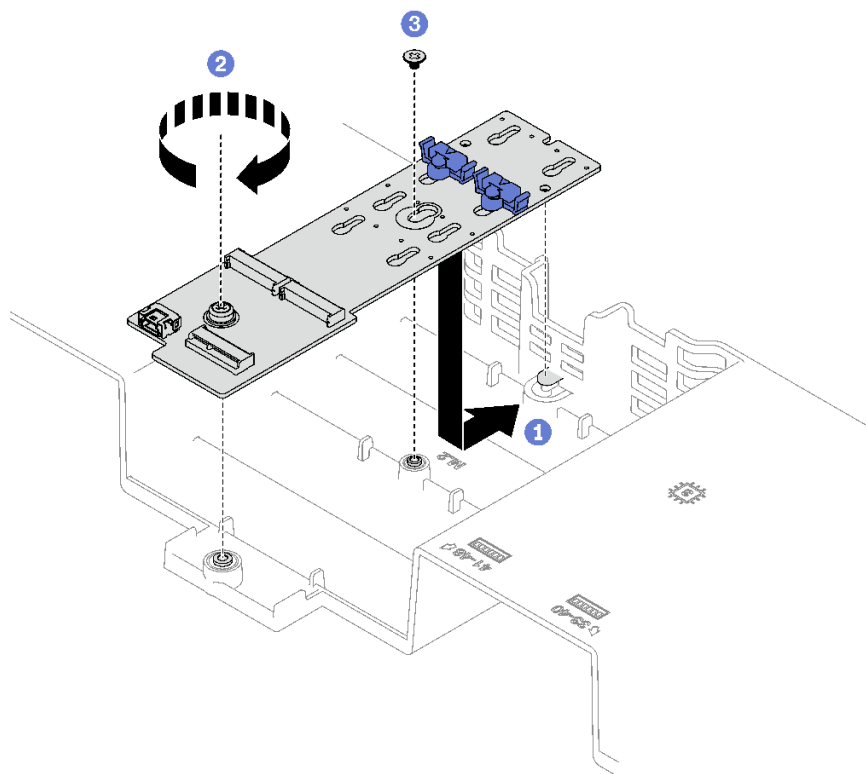
圖例 81. M.2 背板安裝
