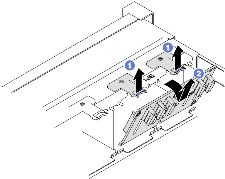
圖例 26. 卸下 2.5 吋硬碟背板
