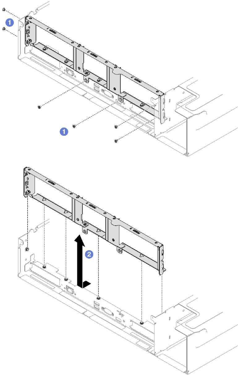
圖例 142. 卸下後壁
