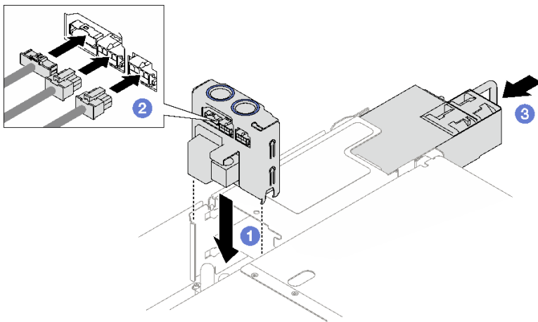
圖例 124. 安裝電源配送板
