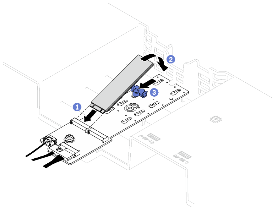
圖例 84. M.2 硬碟安裝
