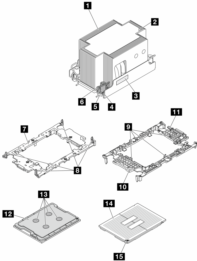
圖例 136. PHM 元件
