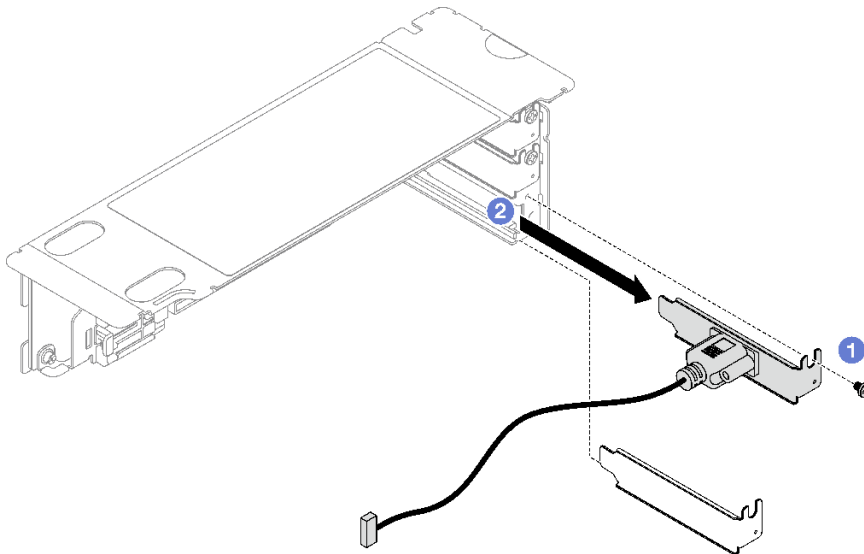
圖例 148. 卸下序列埠模組
