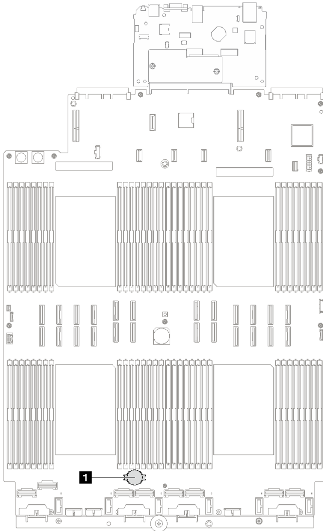
圖例 55. CMOS 電池插槽位置
