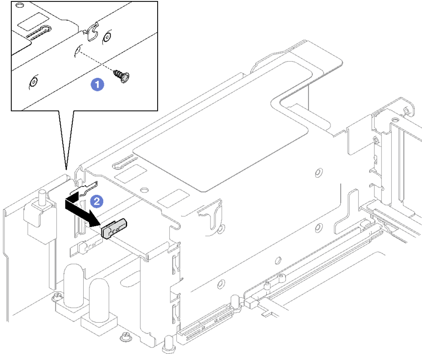
圖例 129. 卸下電源供應器鑰匙
