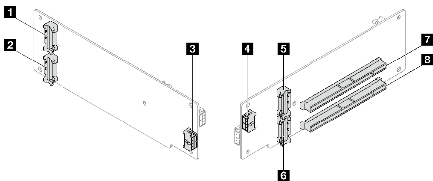
圖例 166. 雙插槽 PCIe Gen5 擴充卡接頭
