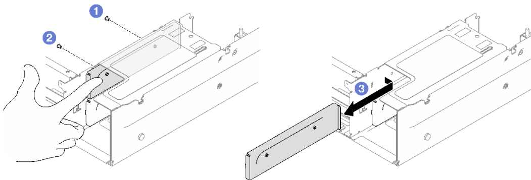
圖例 127. 卸下電源供應器托架
