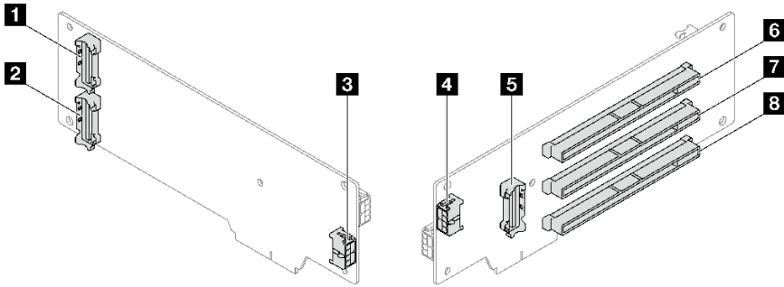
圖例 167. 三插槽 PCIe Gen4 擴充卡接頭 ( 含電源接頭 )
