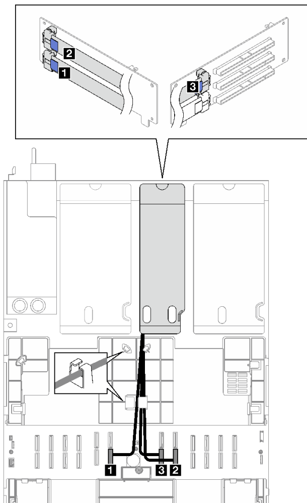
圖例 188. 三插槽 PCIe 擴充卡 2 (含序列埠模組) 的纜線佈線
