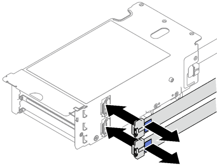
圖例 108. 拔除纜線
