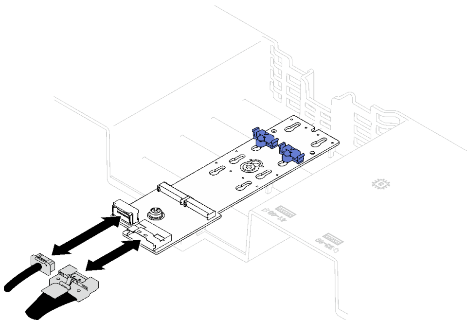
圖例 78. 拔除 SATA/x4 NVMe M.2 背板纜線
