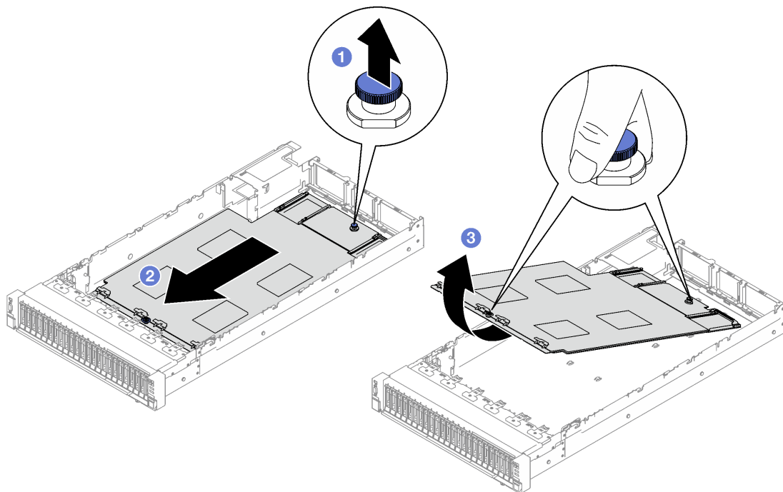
圖例 154. 卸下主機板組件
