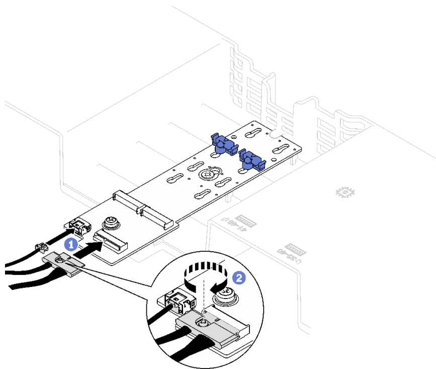
圖例 79. SATA/NVMe 或 NVMe M.2 背板纜線連接
