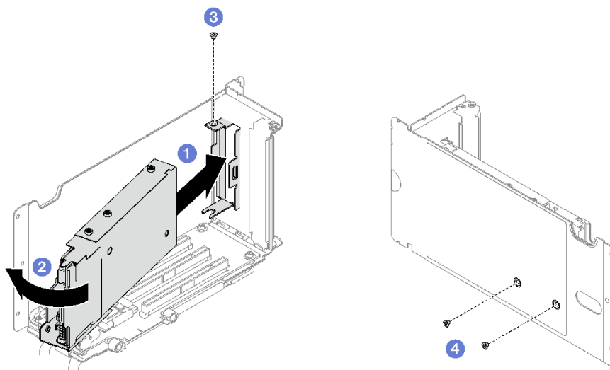
圖例 34. 安裝 7 公釐框架
