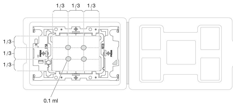
圖例 138. 運送匣中的處理器塗上散熱膏
