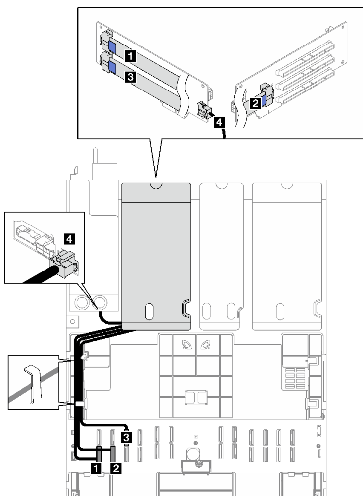
圖例 190. 三插槽 PCIe 擴充卡 3 的纜線佈線
