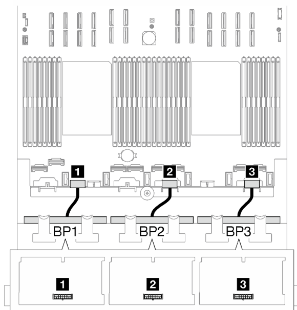
圖例 173. 2.5 吋硬碟背板的電源線纜線佈線
