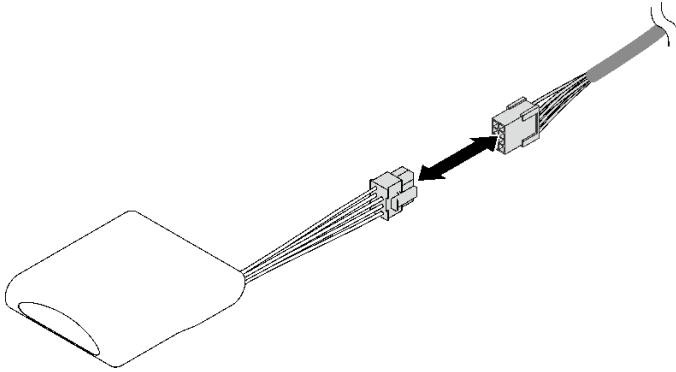
圖例 36. 拔掉快閃記憶體電源模組纜線
