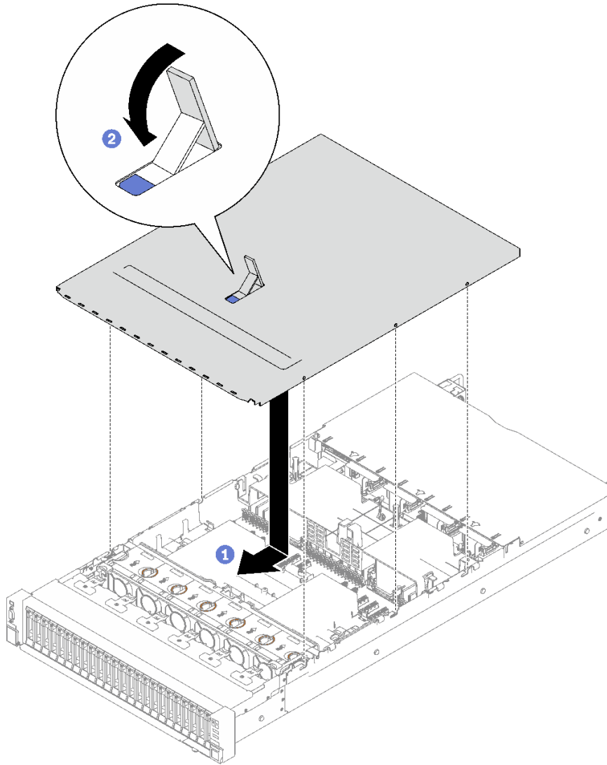
圖例 162. 安裝前方上蓋
