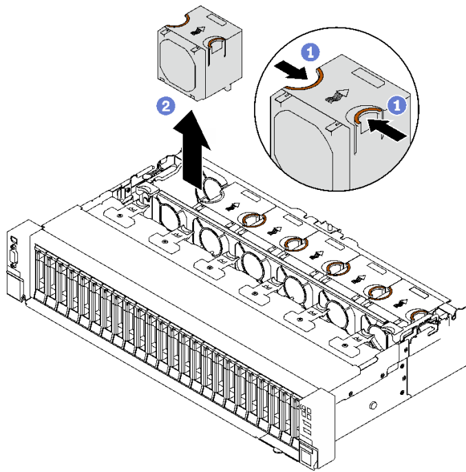
圖例 60. 卸下風扇
