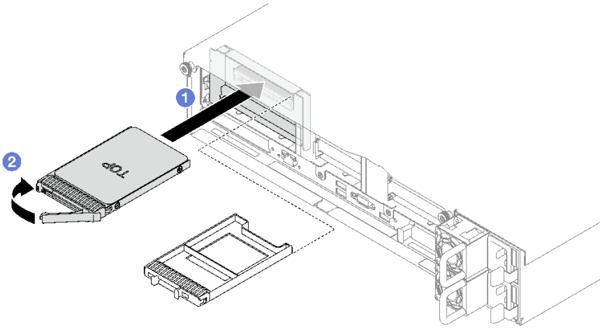
圖例 35. 安裝 7 公釐硬碟
