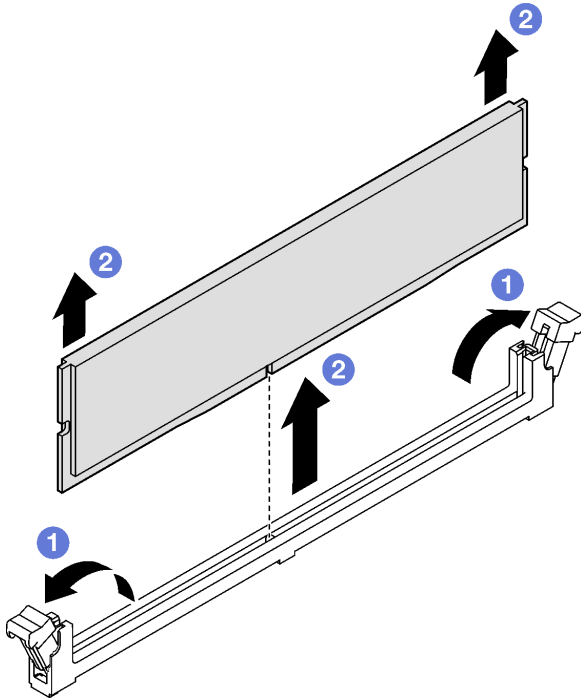
圖例 88. 卸下記憶體模組
