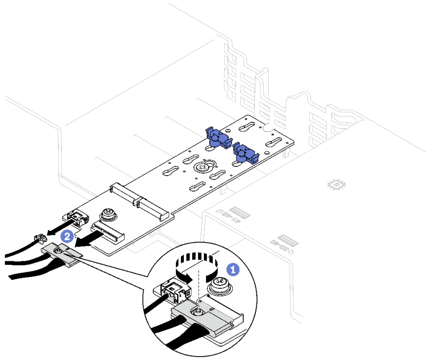
圖例 45. 拔除 SATA/NVMe M.2 背板纜線
