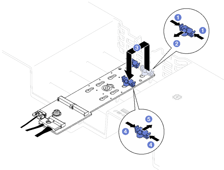
圖例 82. M.2 背板固定器調整
