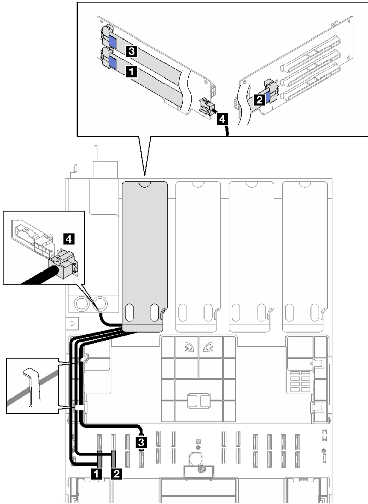
圖例 195. PCIe 擴充卡 D 的纜線佈線
