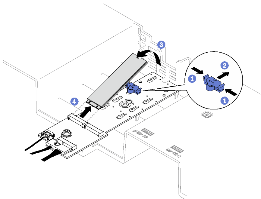
圖例 75. 卸下 M.2 硬碟
