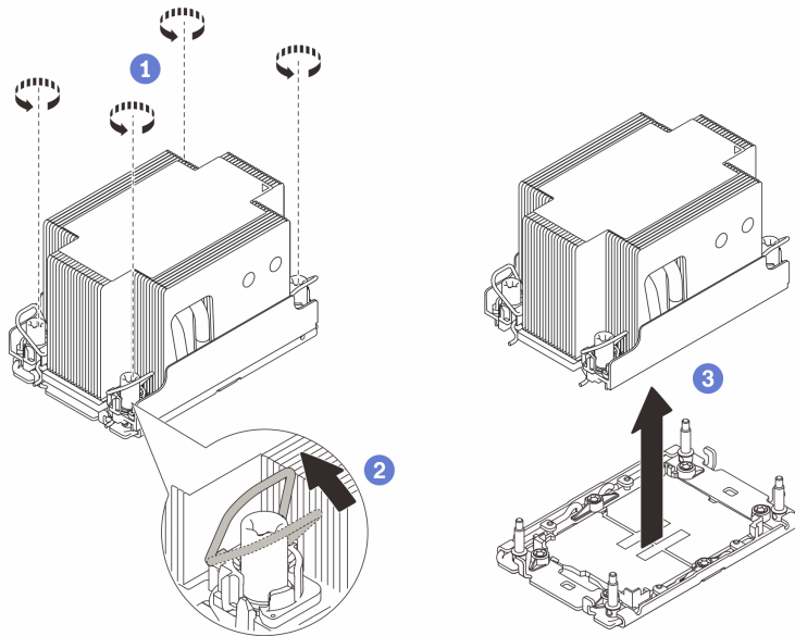
圖例 132. 卸下 2U 標準 PHM
