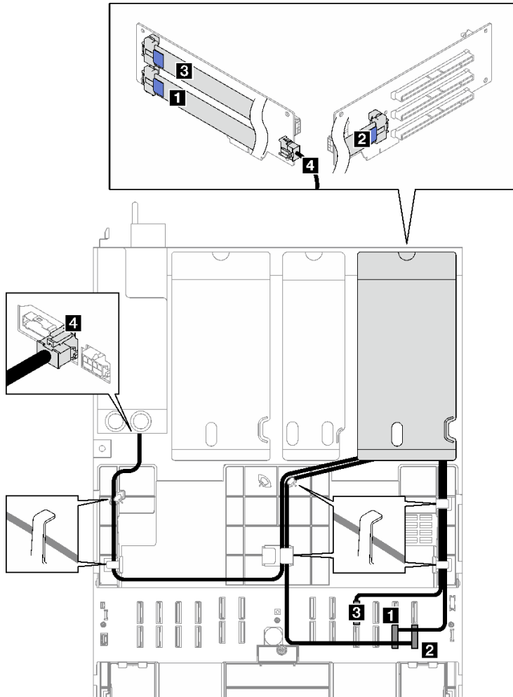
圖例 185. 三插槽 PCIe HL 擴充卡 1 的纜線佈線
