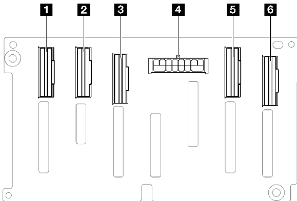
圖例 165. 8x 2.5 吋 SAS/SATA/NVMe 背板接頭
