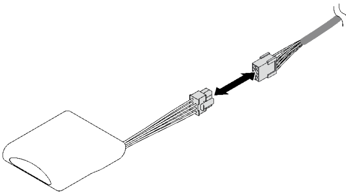
圖例 51. 連接快閃記憶體電源模組纜線
