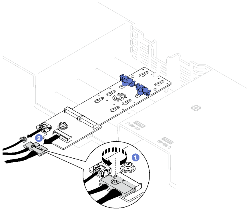
圖例 77. 拔除 SATA/NVMe 或 NVMe M.2 背板纜線
