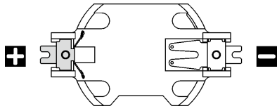
圖例 53. CMOS 電池的正 (+) 極和負 (-) 極
