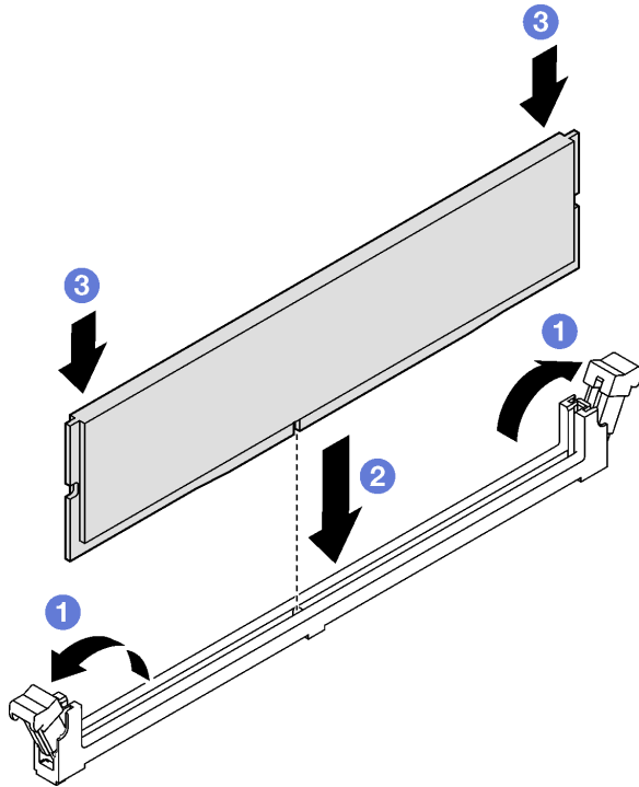
圖例 90. 安裝記憶體模組
