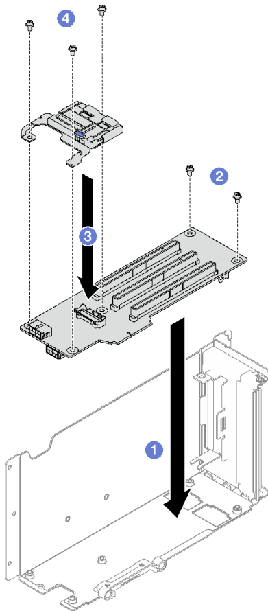
圖例 117. 安裝 PCIe 擴充卡
