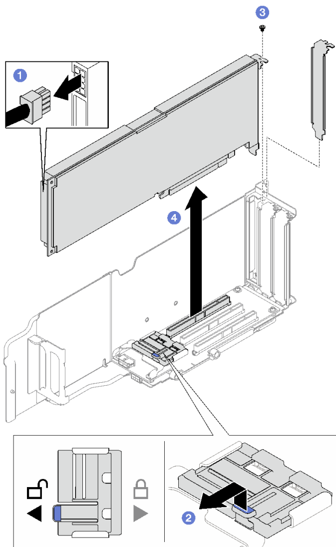
圖例 69. 卸下單寬 GPU 配接卡
