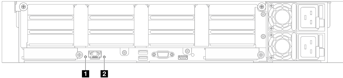
圖例 203. 背面圖上的系統 LED - 配備四個 PCIe 擴充卡的伺服器型號
