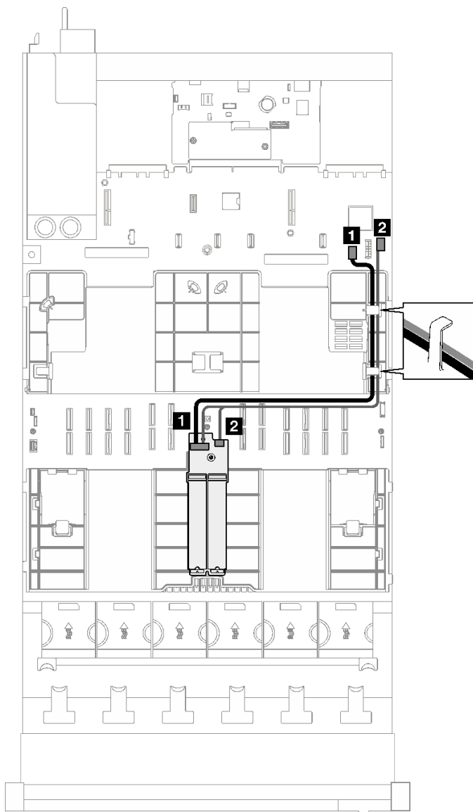
圖例 178. SATA/x4 NVMe M.2 背板至 PCH 的纜線佈線
