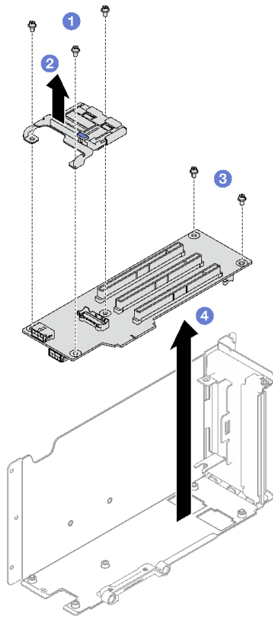
圖例 110. 卸下 PCIe 擴充卡
