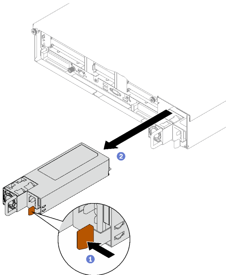
圖例 125. 電源供應器卸下
