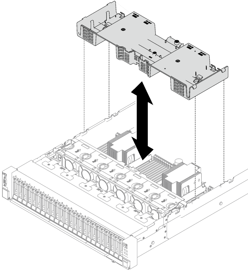
圖例 39. 卸下前方空氣擋板
