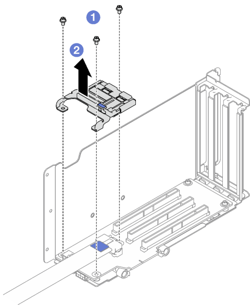
圖例 118. 卸下 PCIe 固定器
