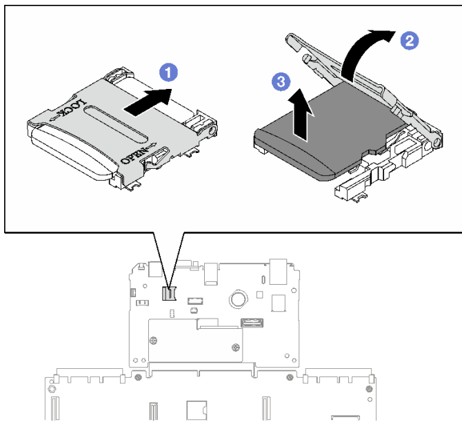
圖例 91. 卸下 MicroSD 卡
