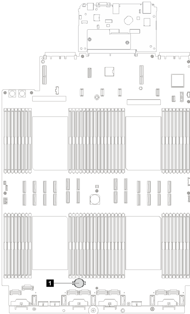
圖例 52. CMOS 電池位置
