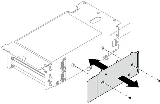
圖例 113. 卸下纜線蓋
