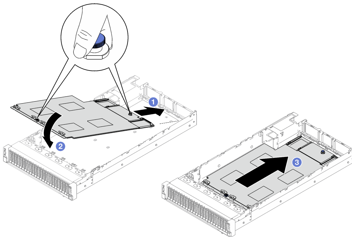
圖例 157. 安裝主機板組件
