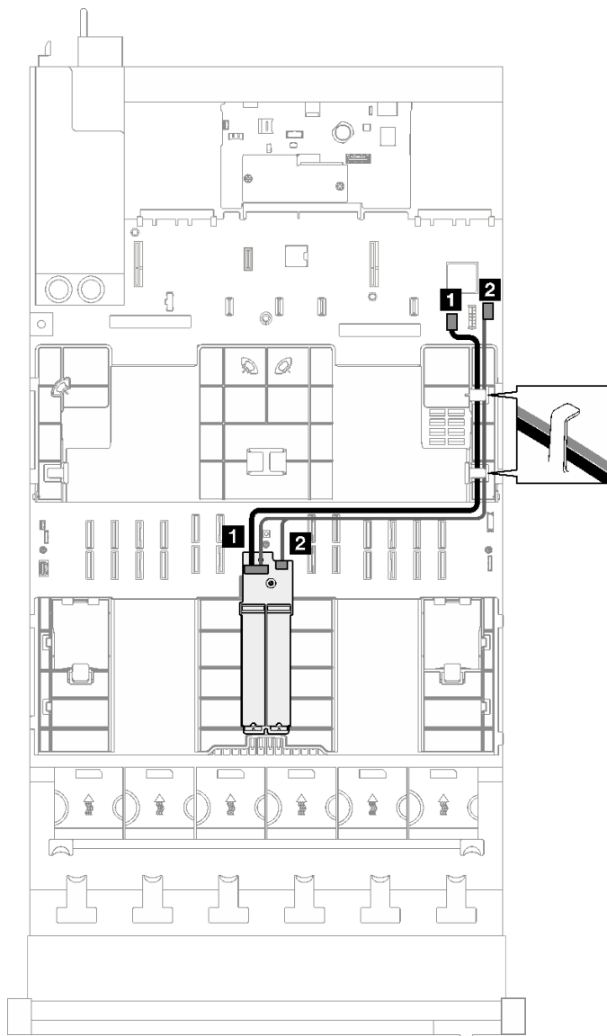
圖例 177. SATA/NVMe 或 NVMe M.2 背板的纜線佈線
