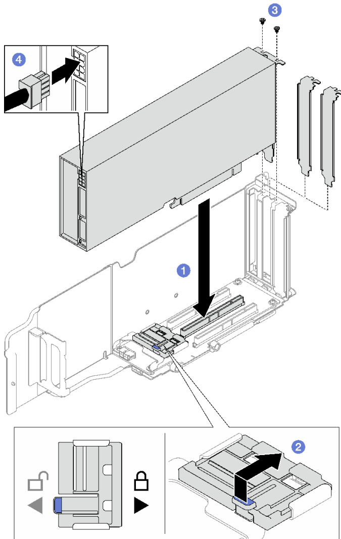
圖例 72. 安裝雙寬 GPU 配接卡
