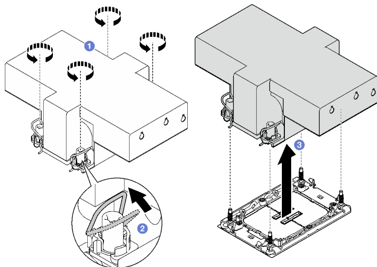
圖例 133. 卸下 2U 效能 PHM
