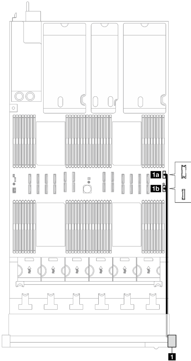
圖例 176. 正面 I/O 模組的纜線佈線
