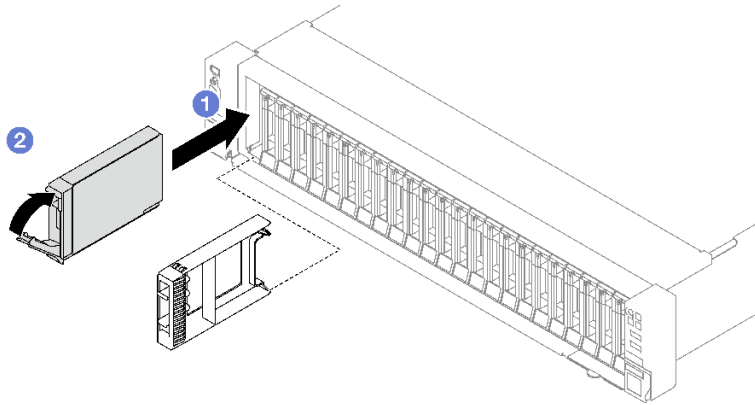
圖例 29. 安裝 2.5 吋熱抽換硬碟
