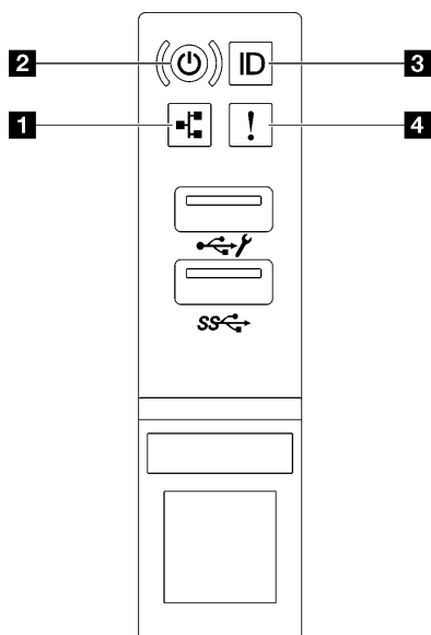
圖例 199. 正面 I/O 模組 LED
