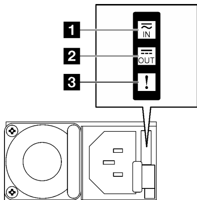
圖例 200. CFFv4 電源供應器 LED
