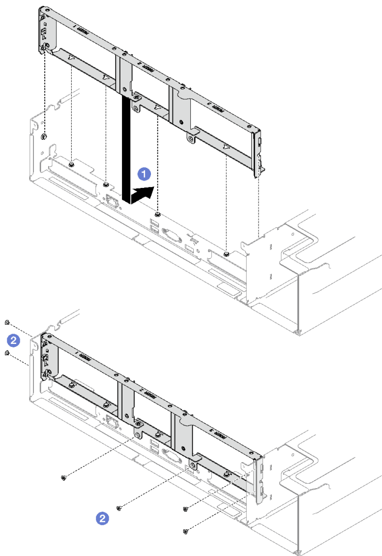
圖例 143. 後壁安裝
