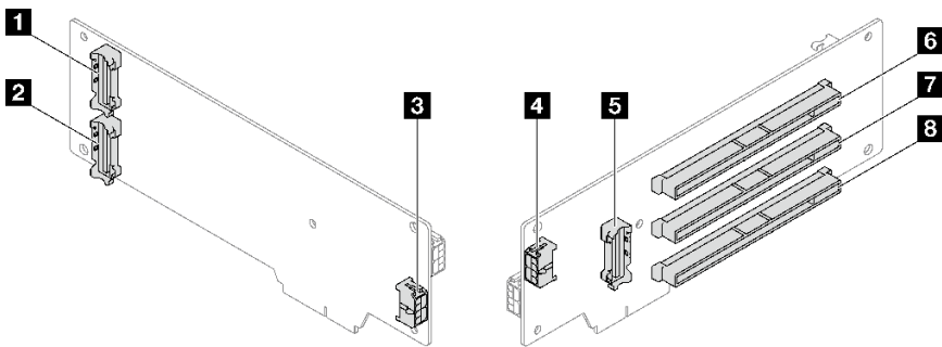
圖例 168. 三插槽 PCIe Gen5 擴充卡接頭 ( 含電源接頭 )
