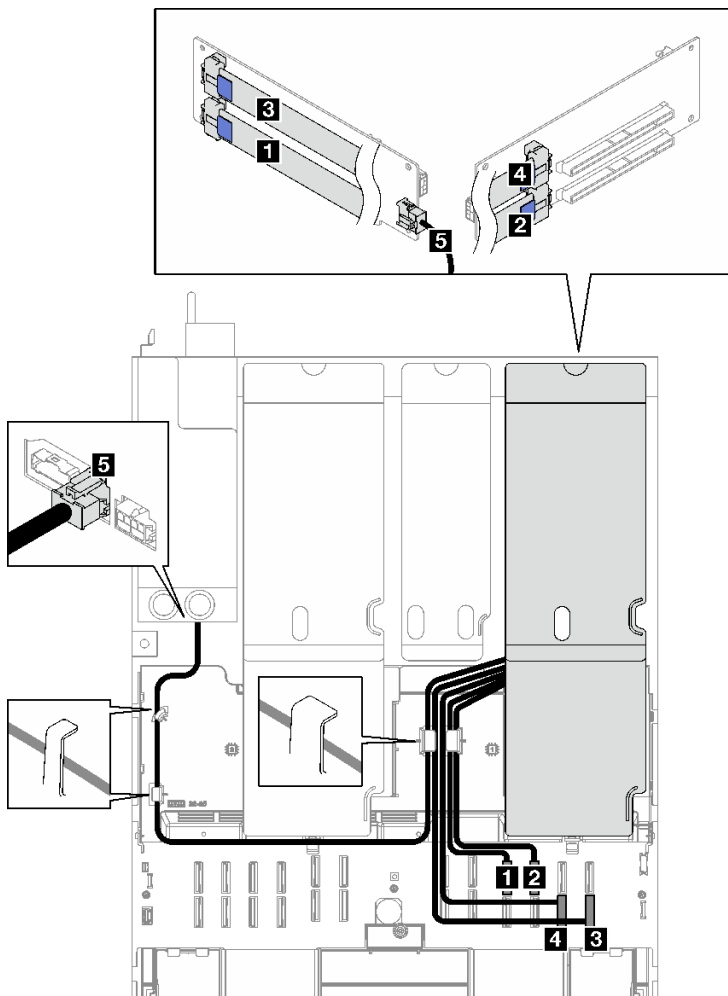
圖例 182. 雙插槽 PCIe FL 擴充卡 1 的纜線佈線
