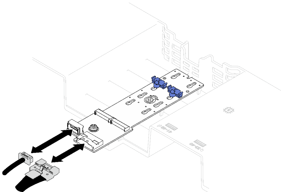
圖例 42. 連接 SATA/x4 NVMe M.2 背板纜線
