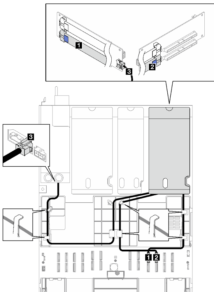
圖例 183. 雙插槽 PCIe HL 擴充卡 1 ( 含 7 公釐框架 ) 的纜線佈線
