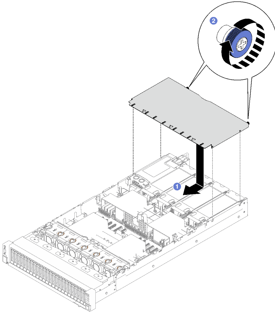
圖例 161. 安裝後方上蓋
