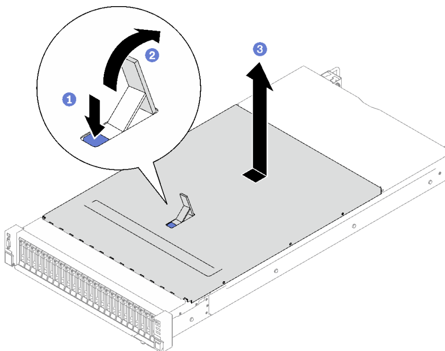
圖例 159. 卸下前方上蓋
