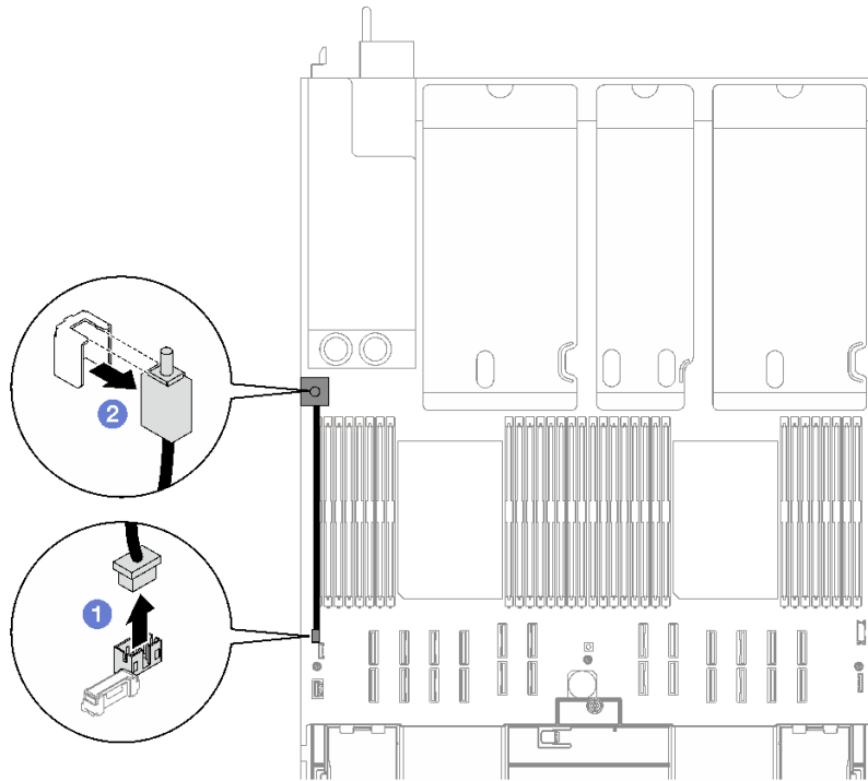
圖例 73. 卸下入侵開關
