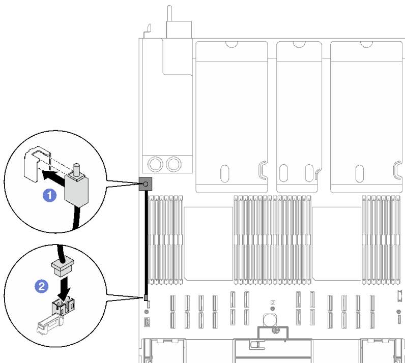
圖例 74. 入侵開關安裝
