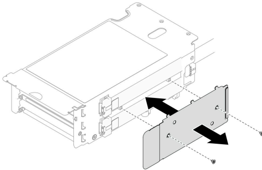
圖例 116. 安裝纜線蓋
