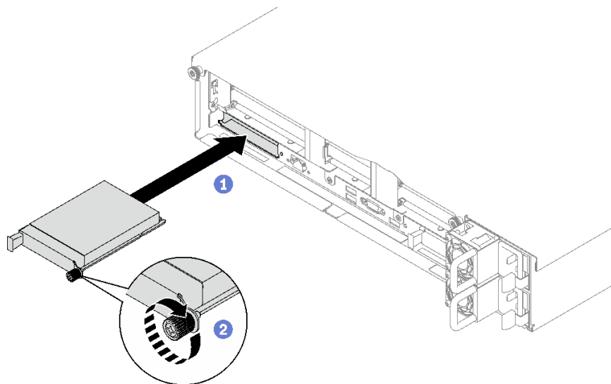
圖例 94. OCP 模組安裝
