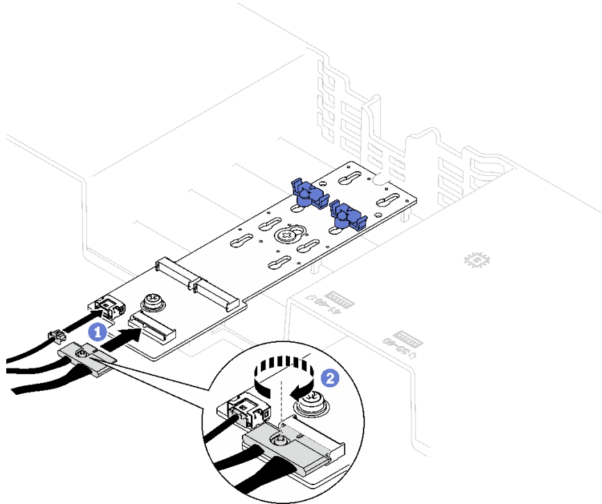
圖例 49. 連接 SATA/NVMe M.2 背板纜線
