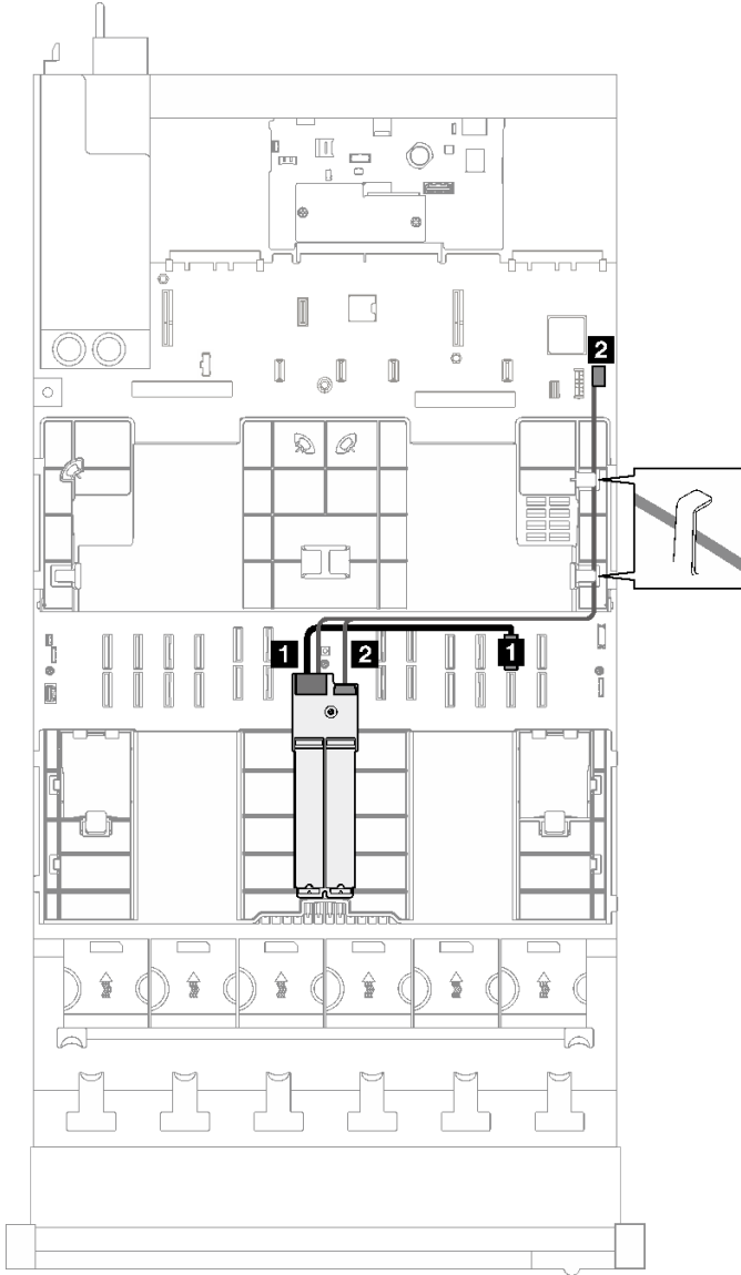
圖例 179. SATA/x4 NVMe M.2 背板至處理器的纜線佈線
