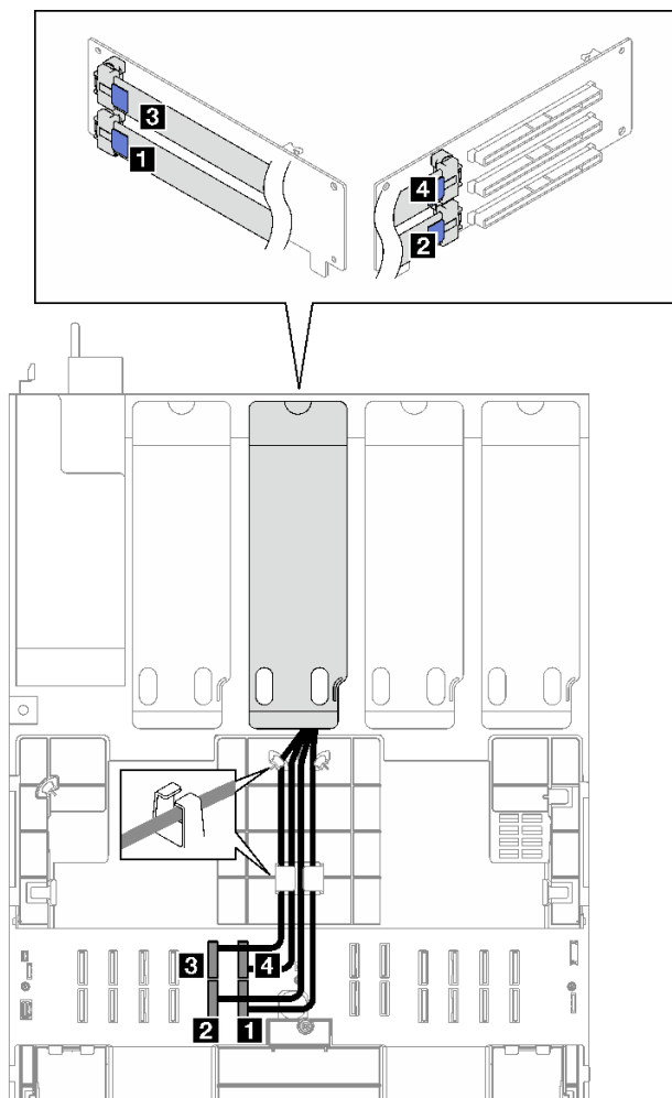
圖例 193. PCIe 擴充卡 C 的纜線佈線
