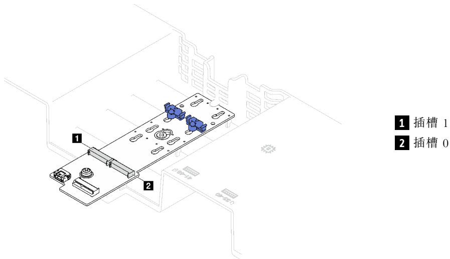
圖例 83. M.2 硬碟插槽
