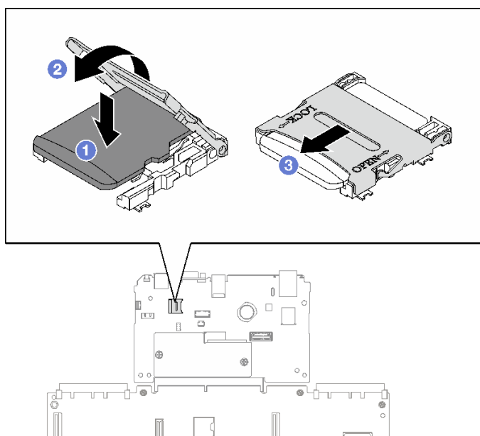
圖例 92. 安裝 MicroSD 卡
