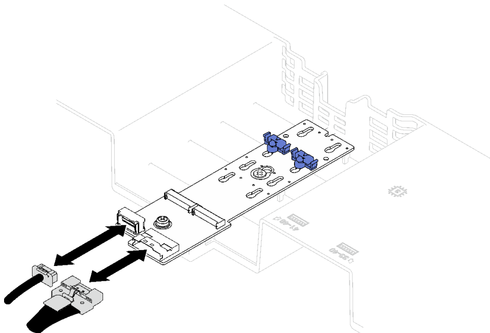
圖例 46. 拔除 SATA/x4 NVMe M.2 背板纜線
