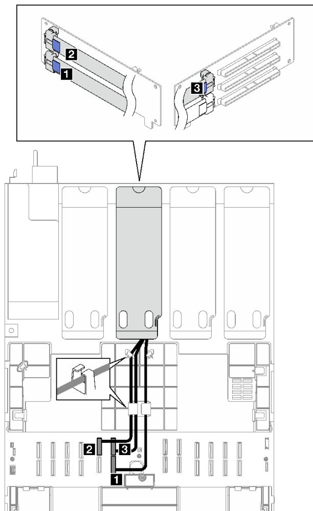
圖例 194. PCIe 擴充卡 C (含序列埠模組) 的纜線佈線
