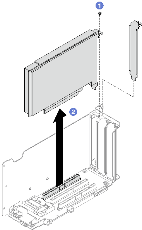
圖例 99. 卸下 PCIe 配接卡
