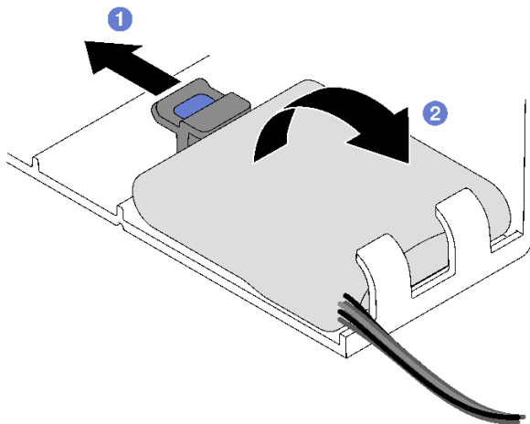
圖例 65. 卸下快閃記憶體電源模組
