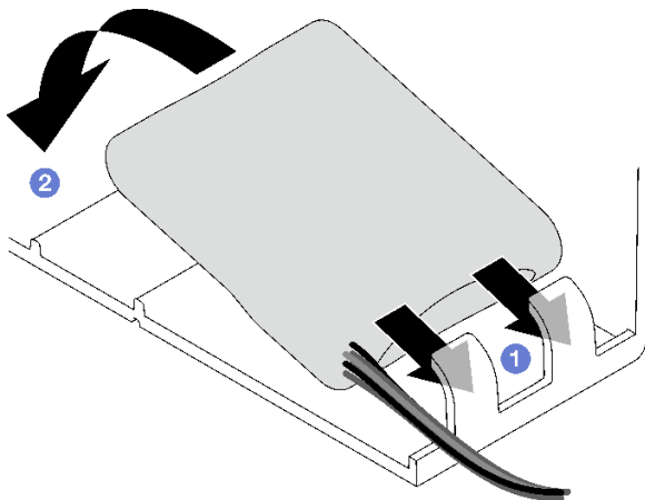
圖例 67. 快閃記憶體電源模組安裝
