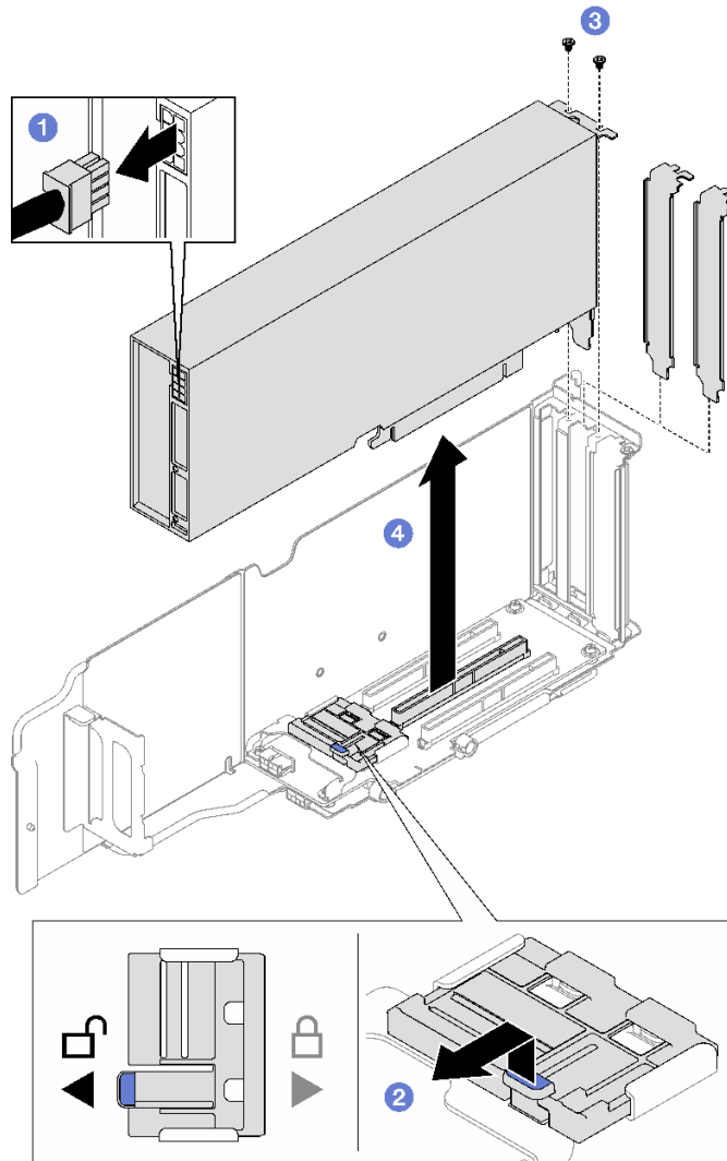
圖例 70. 卸下雙寬 GPU 配接卡
