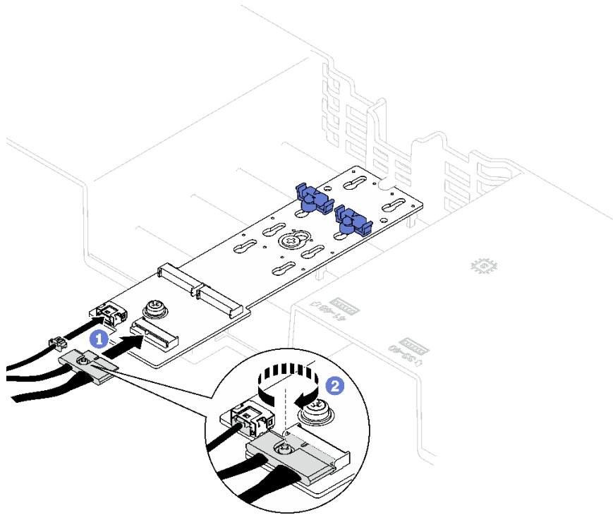
圖例 41. 連接 SATA/NVMe M.2 背板纜線
