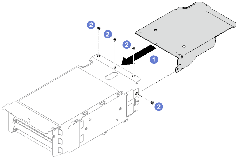
圖例 121. 安裝 PCIe 擴充卡延伸器
