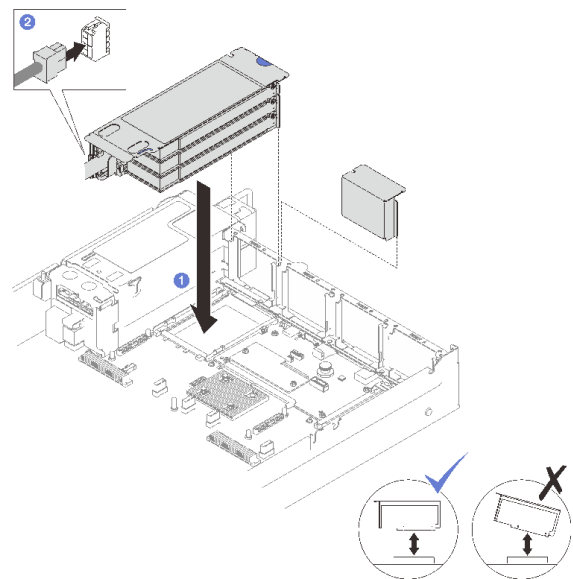
圖例 104. 安裝 PCIe LP 擴充卡（含電源線）
