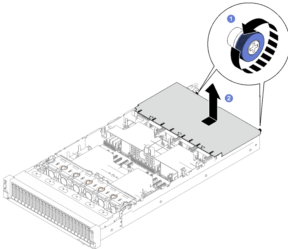
圖例 160. 卸下後方上蓋
