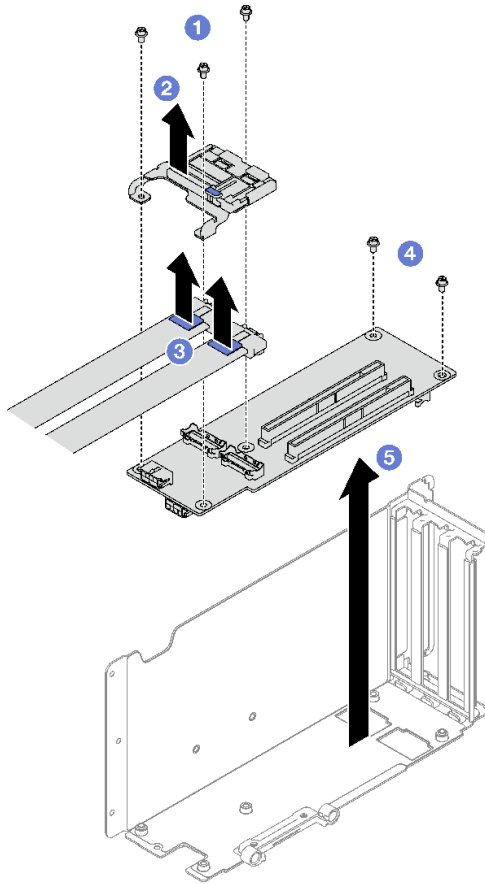
圖例 109. 卸下 PCIe 擴充卡
