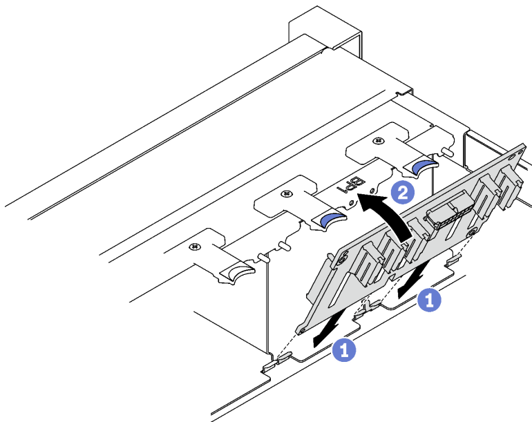
圖例 28. 2.5 吋硬碟背板安裝
