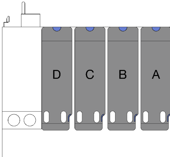
圖例 102. 配備四個 PCIe 擴充卡之伺服器型號的 PCIe 擴充卡類型和位置
