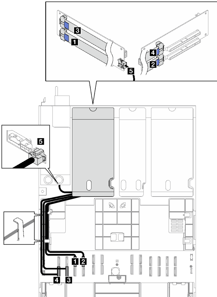
圖例 189. 雙插槽 PCIe 擴充卡 3 的纜線佈線
