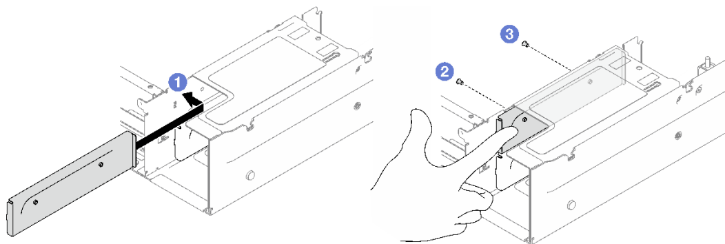
圖例 128. 安裝電源供應器托架
