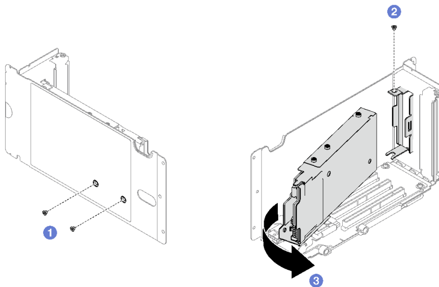
圖例 31. 卸下 7 公釐框架
