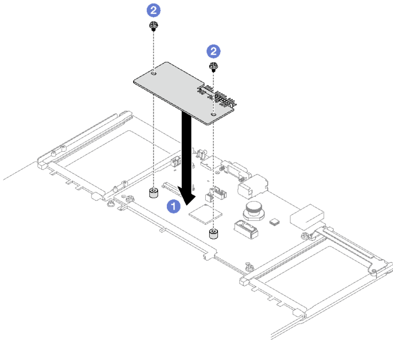
圖例 153. 安裝韌體和 RoT 安全模組
