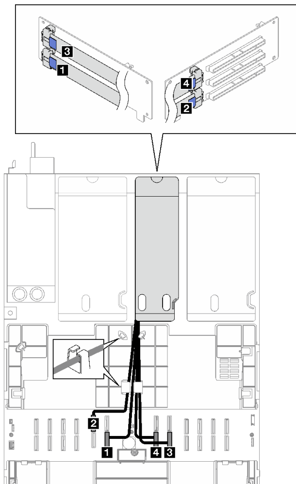
圖例 187. 三插槽 PCIe 擴充卡 2 的纜線佈線
