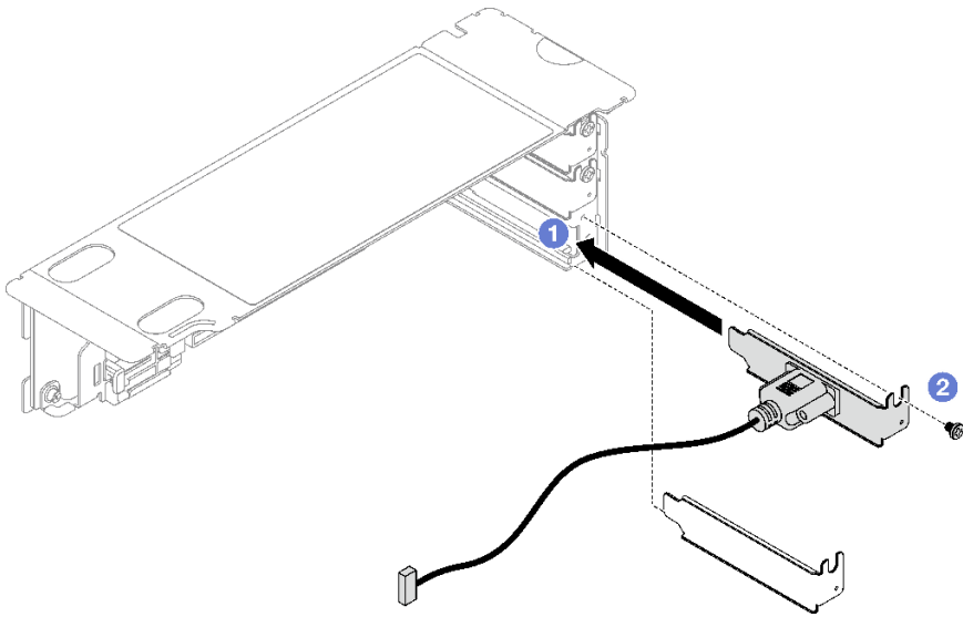
圖例 149. 序列埠模組安裝
