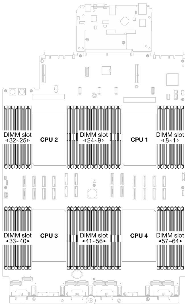
圖例 87. 記憶體模組和處理器佈置
