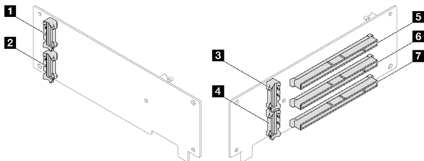
圖例 170. 三插槽 PCIe Gen5 擴充卡接頭 ( 不含電源接頭 )
