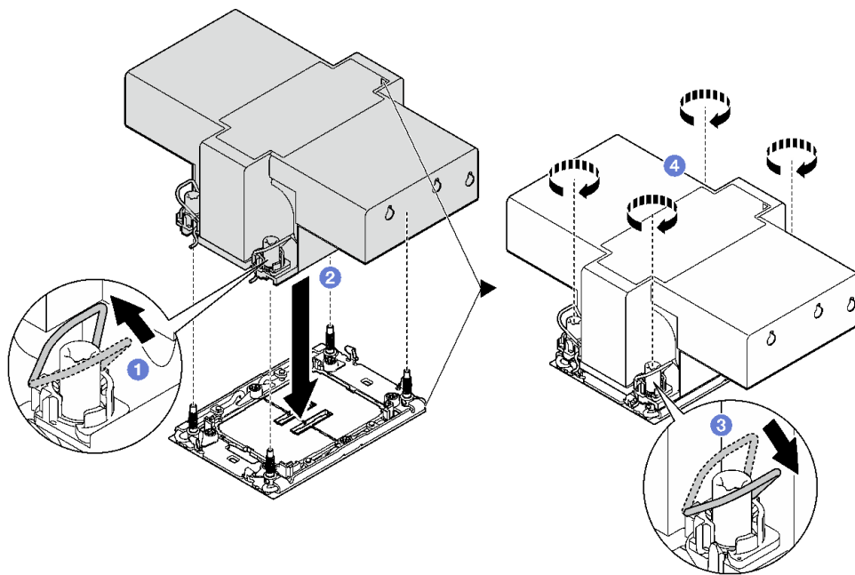
圖例 141. 2U 效能 PHM 安裝
