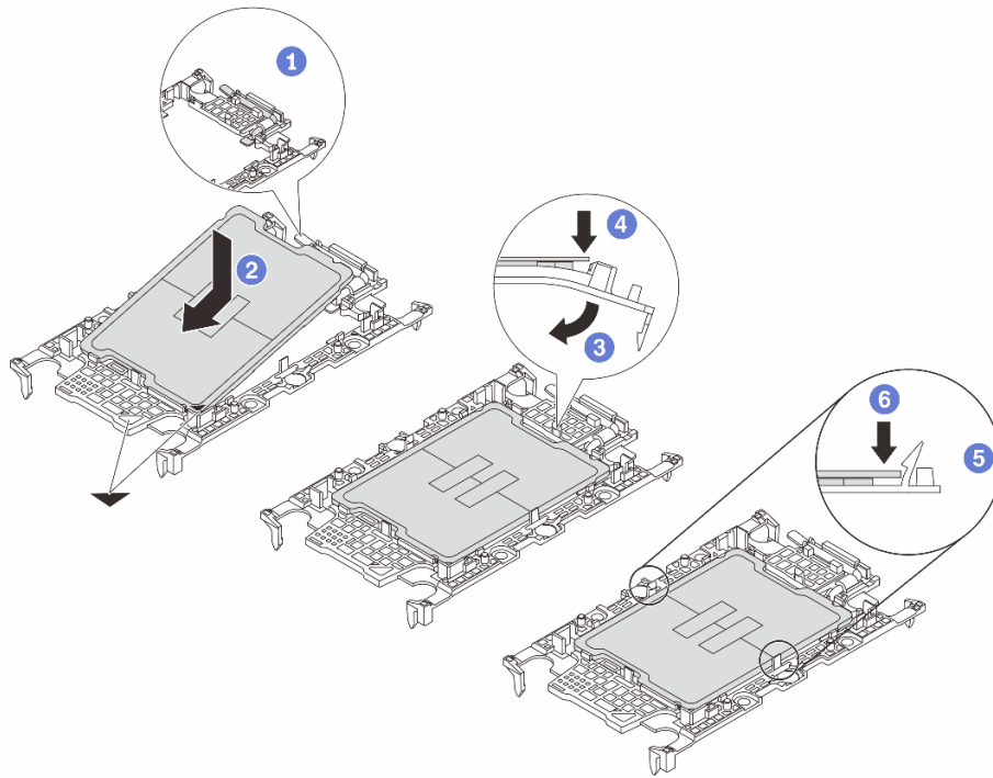
圖例 137. 安裝處理器支架
