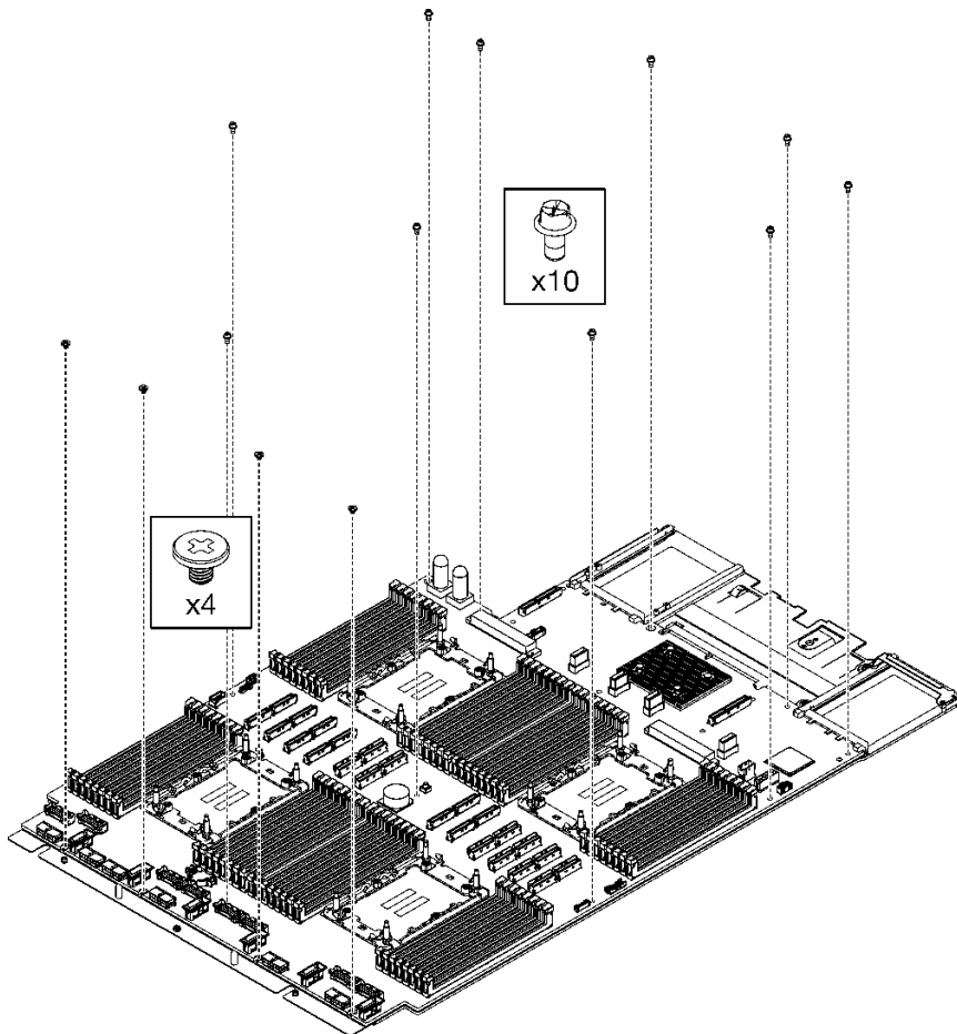
圖例 209. 卸下螺絲
