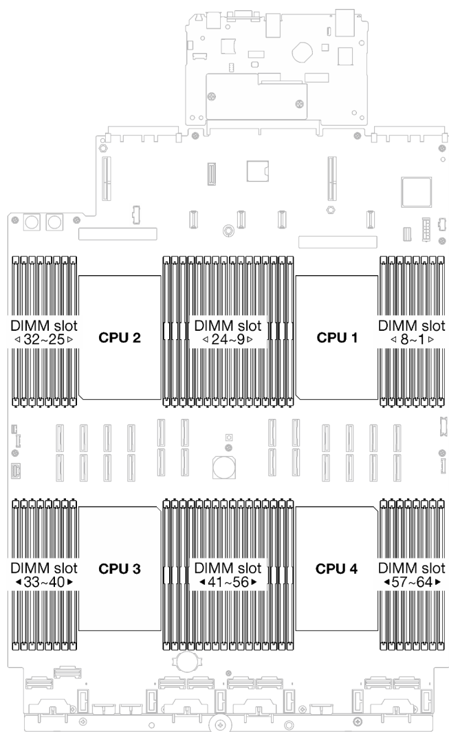
圖例 23. 記憶體模組和處理器佈置
