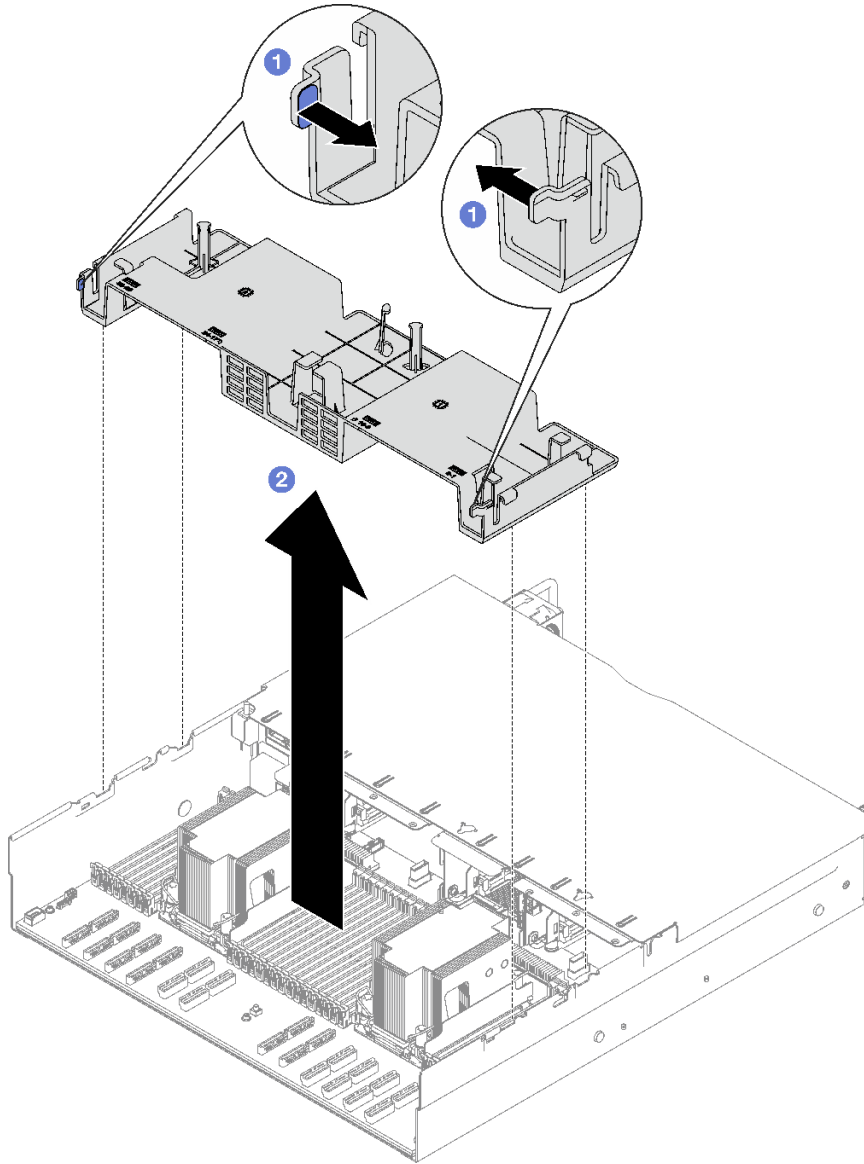
圖例 47. 卸下後方空氣擋板
