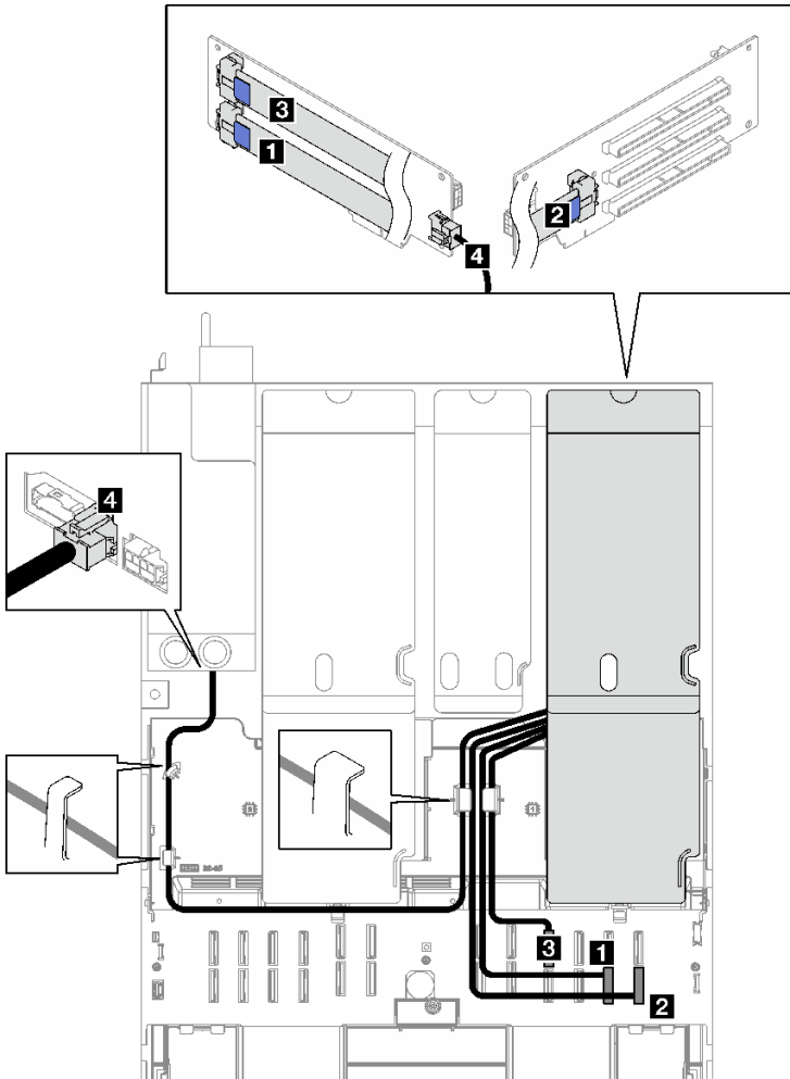
圖例 186. 三插槽 PCIe FL 擴充卡 1 的纜線佈線
