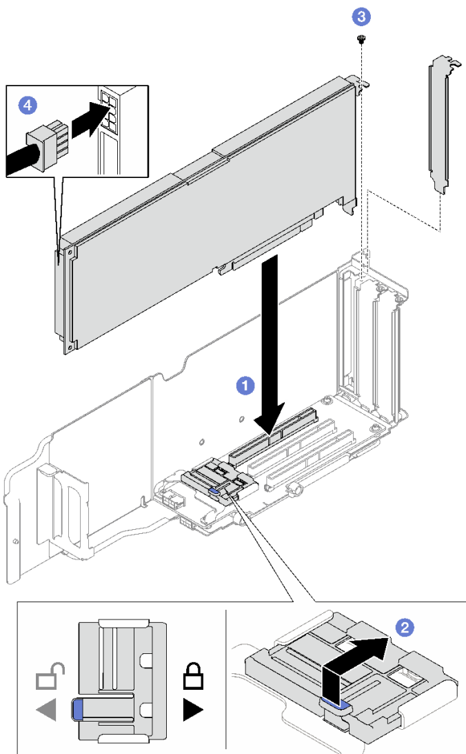
圖例 71. 安裝單寬 GPU 配接卡
