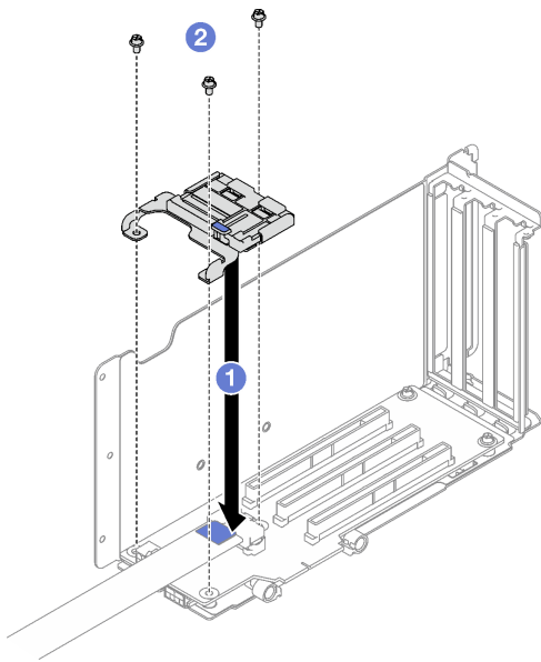
圖例 119. 安裝 PCIe 固定器
