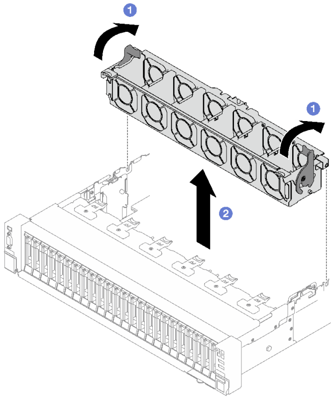
圖例 61. 卸下風扇機盒
