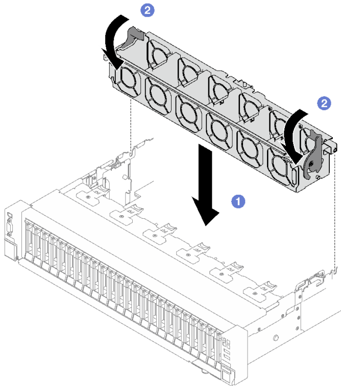
圖例 62. 安裝風扇機盒
