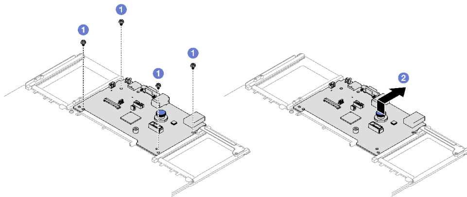
圖例 155. 卸下系統 I/O 板
