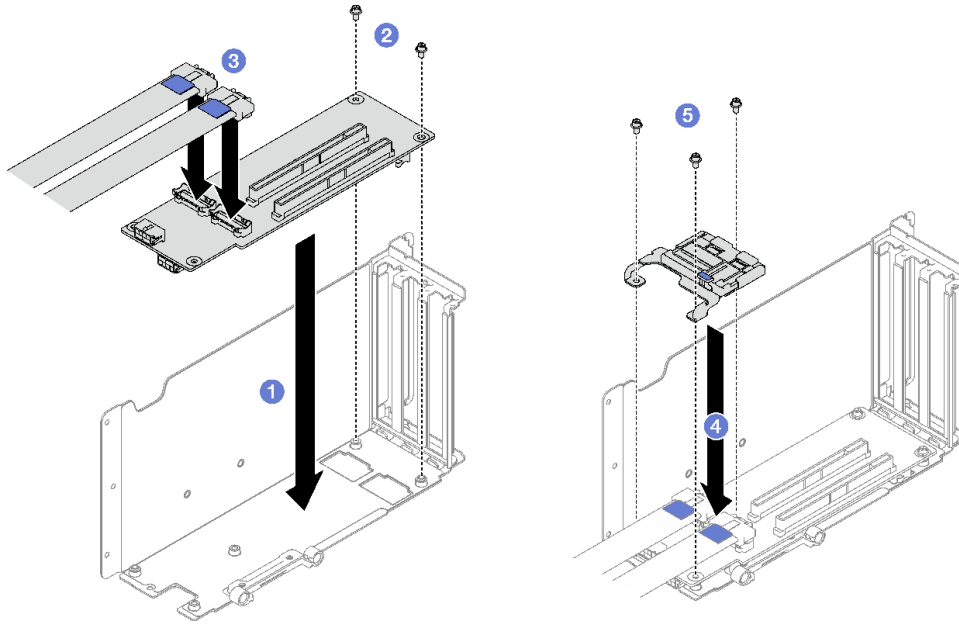
圖例 114. 安裝 PCIe 擴充卡
