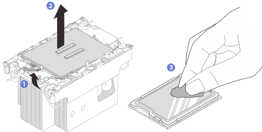
図 212. プロセッサをキャリアとヒートシンクから取り外す
