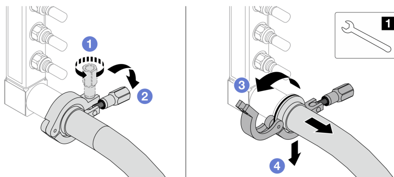
図 137. 接続セットからの多岐管の分離
