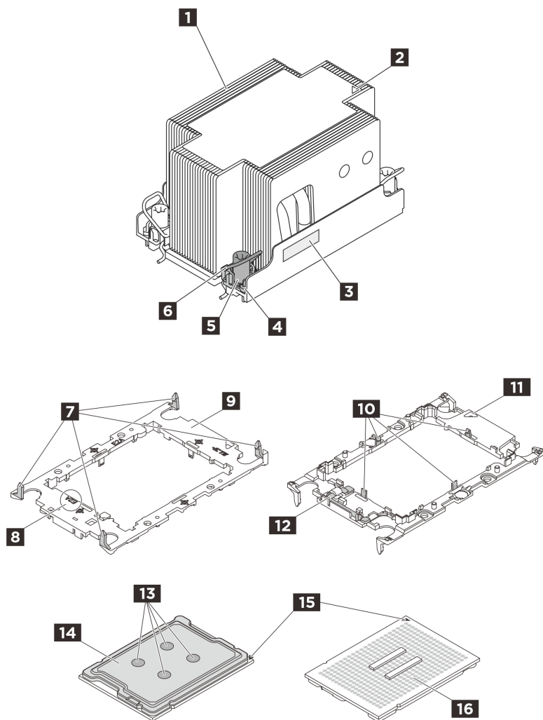
図 209. PHM コンポーネント
