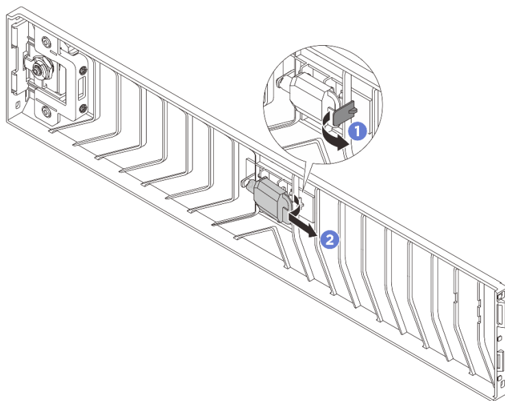
図 234. キーの取り外し
