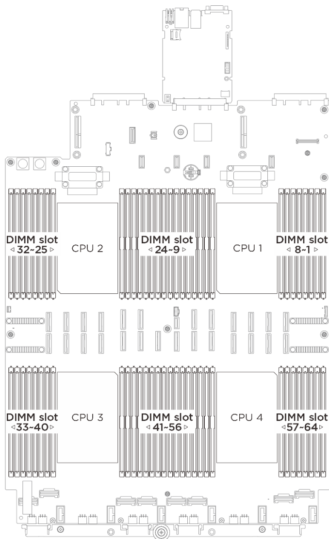
図 171. メモリー・モジュールおよびプロセッサのレイアウト
