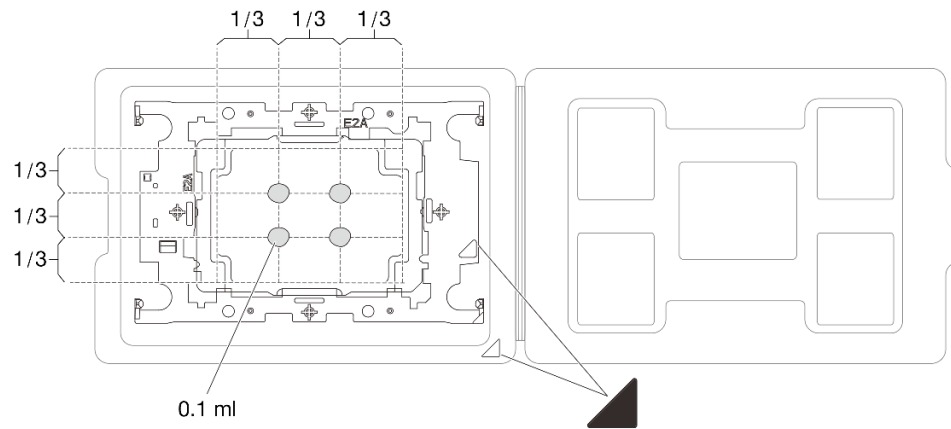
図216. 配送トレイのプロセッサーで熱伝導グリースを塗布する
