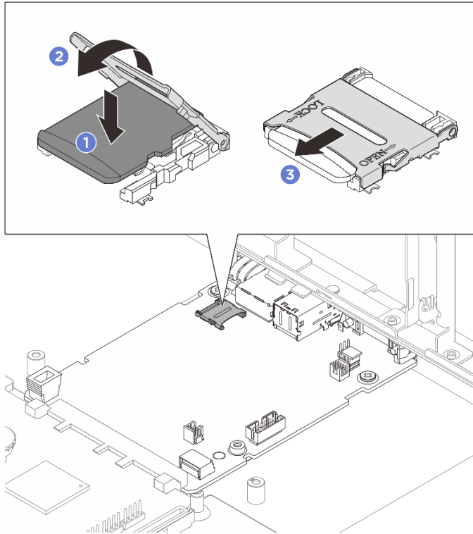
図 176. microSD カードの取り付け
