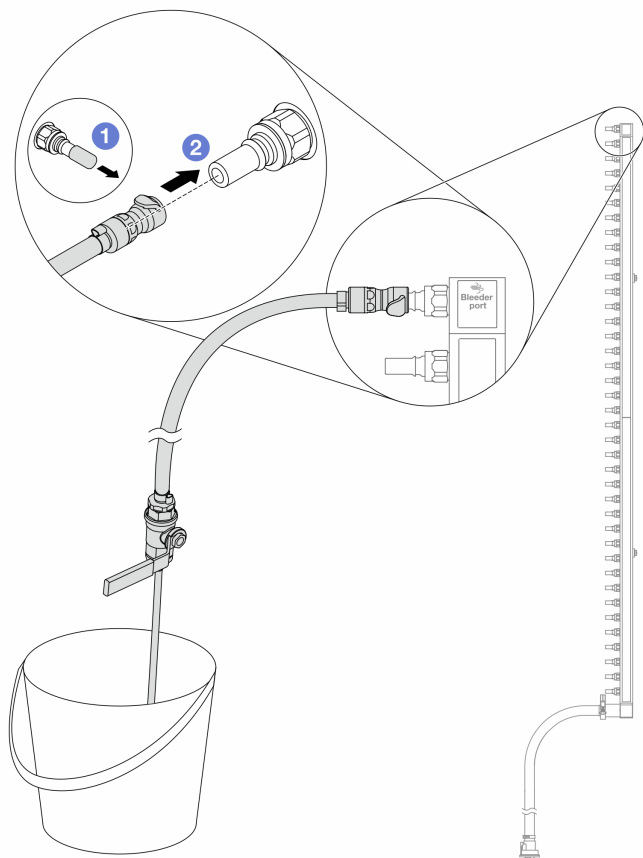
図 157. リターン側へのブリーダー・キットの取り付け
