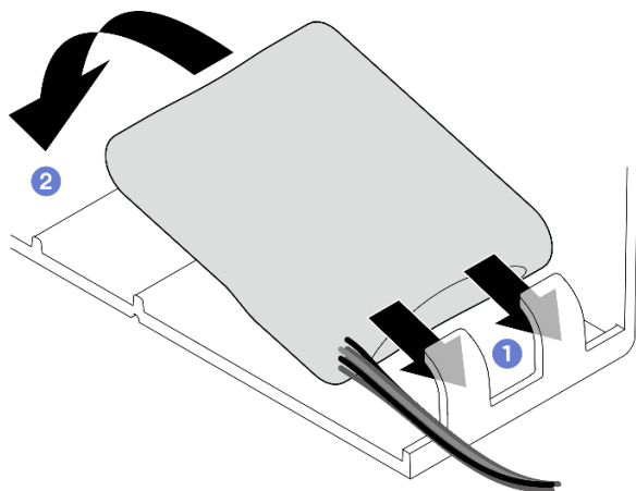
図 75. フラッシュ電源モジュールの取り付け
