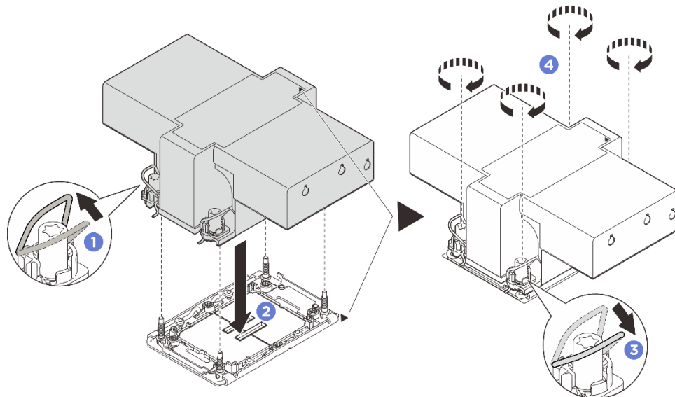
図 219. 2U パフォーマンス PHM の取り付け
