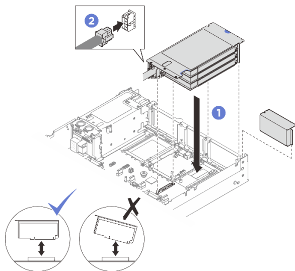
図 191. PCIe FHHL ライザーの取り付け
