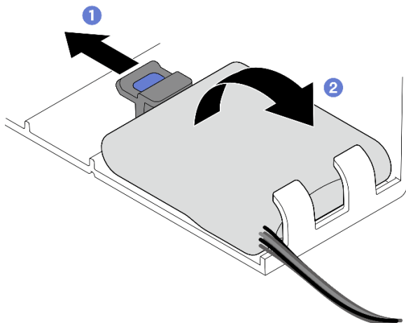
図 73. フラッシュ電源モジュールの取り外し
