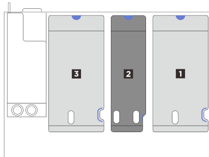
図 179. 3 個の PCIe ライザーを搭載したサーバー・モデル
