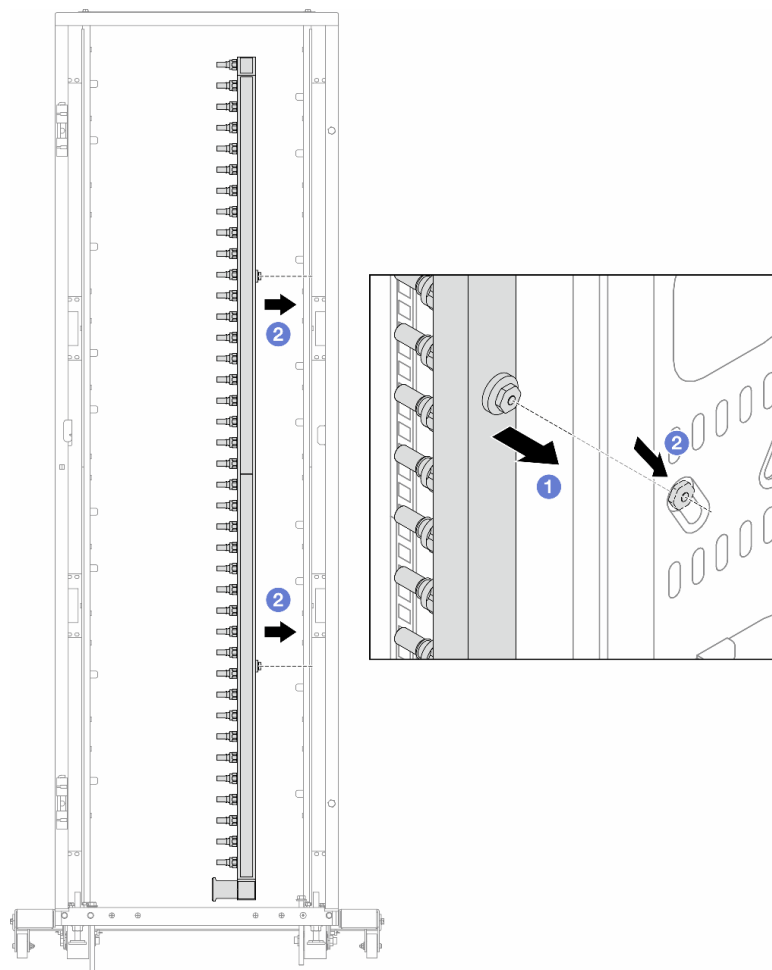
図 138. 多岐管の取り付け
