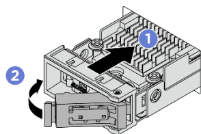
図 93. M.2 ドライブ・アセンブリーの取り付け
