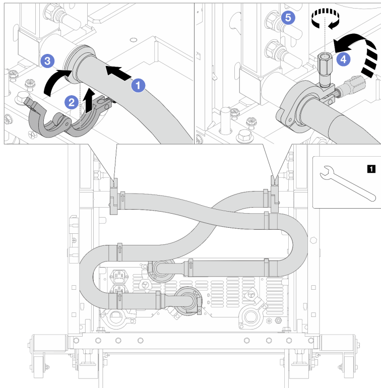
図 141. 接続セットの取り付け
