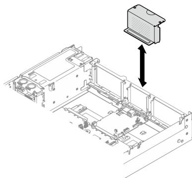
図 97. ライザー・フィラーの取り外し
