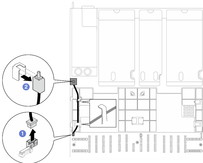
図 94. 侵入検出スイッチの取り外し
