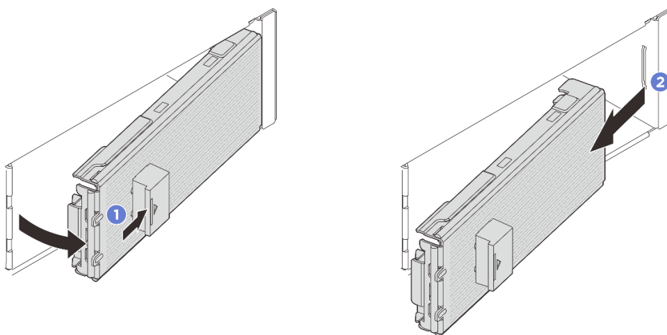
図 56. E3.S ベゼルの取り外し
