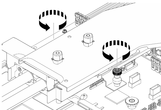
図 102. コールド・プレート・アセンブリの取り外し
