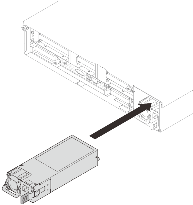
図 208. パワー・サプライ・ユニットの取り付け
