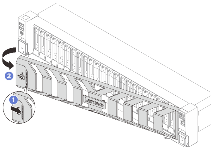
図 233. セキュリティー・ベゼルの取り外し
