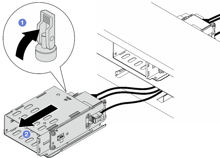
図 52. E3.S 2T ケージの取り外し
