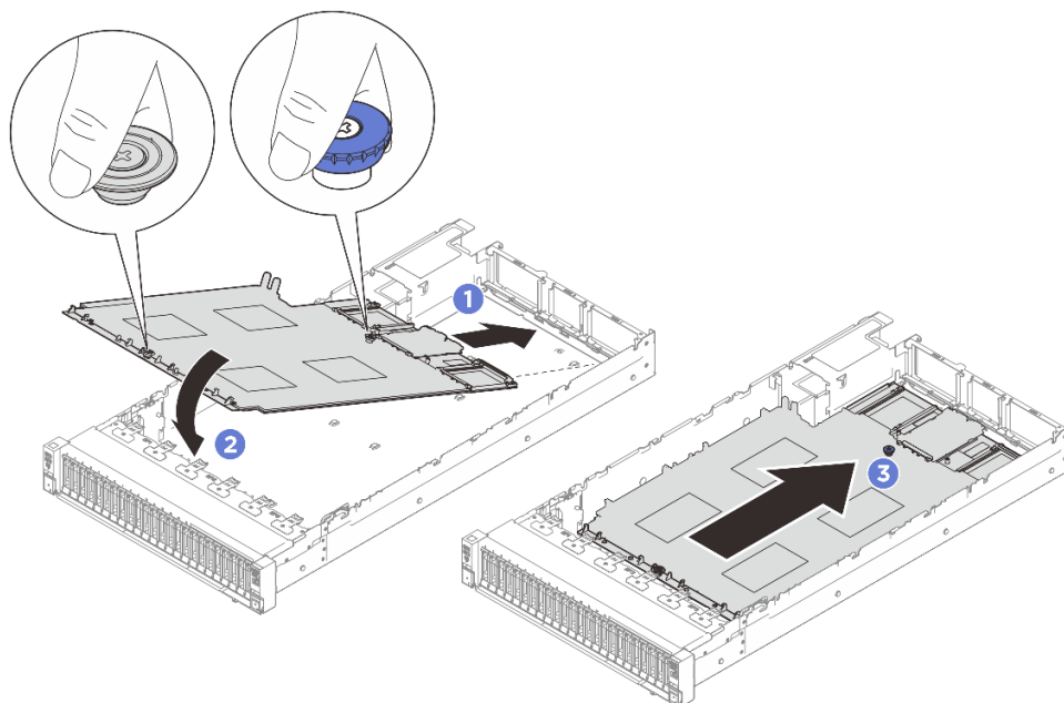
図 246. システム・ボード・アセンブリーの取り付け
