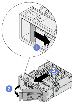
図 82. ホット・スワップ M.2 ドライブ・アセンブリーの取り外し
