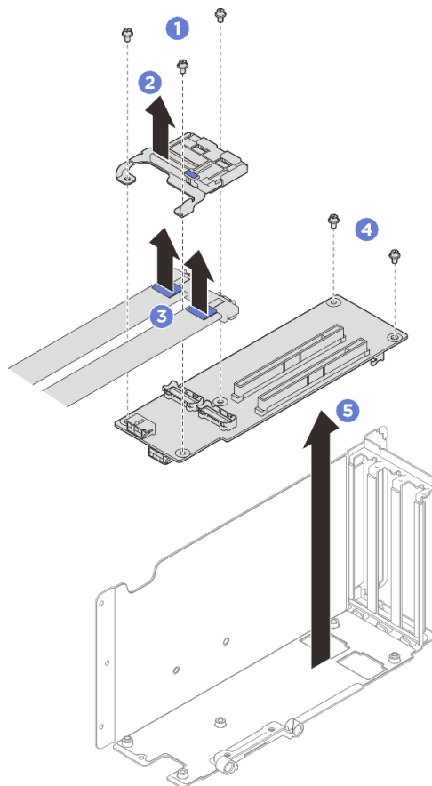
図 195. PCIe ライザー・カードの取り外し
