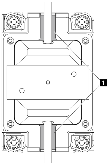
図 275. 漏れやすいエリア
