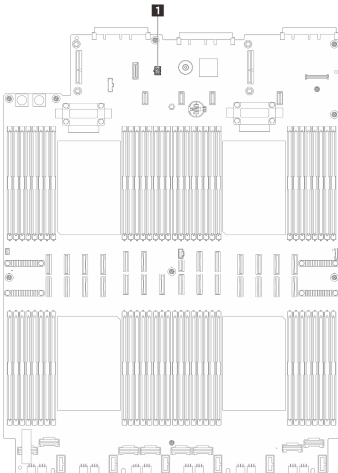
図 114. 漏水検知センサー・モジュールの接続
