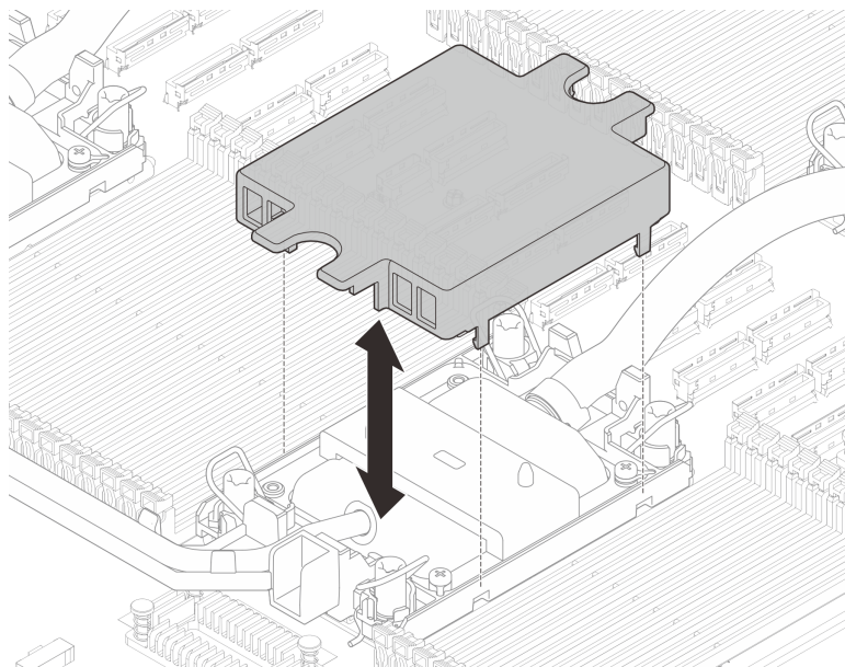
図112. コールド・プレート・カバーの取り付け
