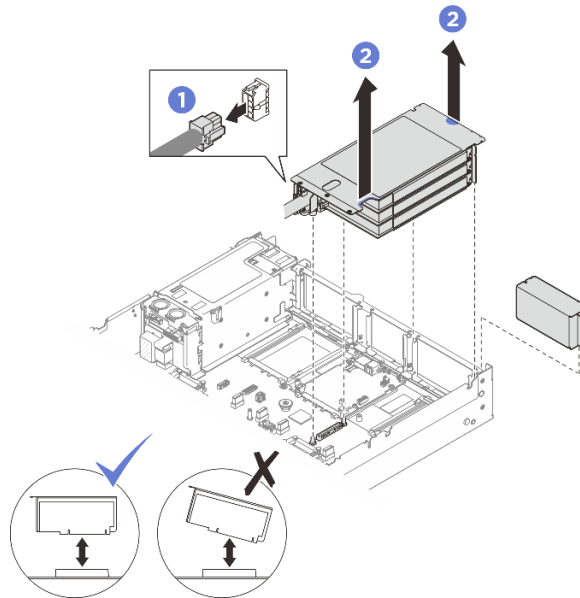
図 183. PCIe FHFL ライザーの取り外し
