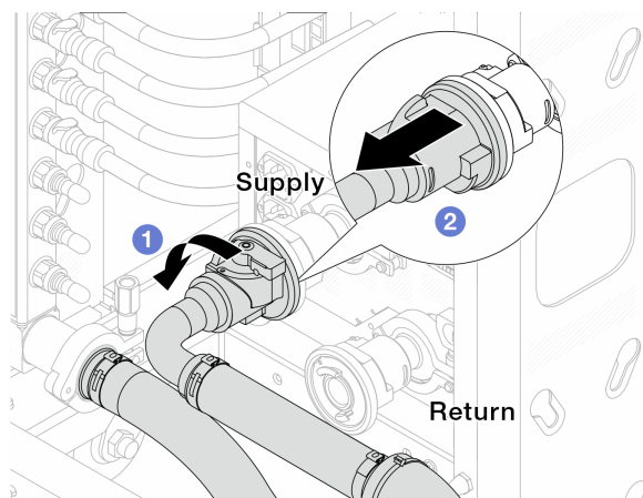
図 131. 接続セットの取り外し
