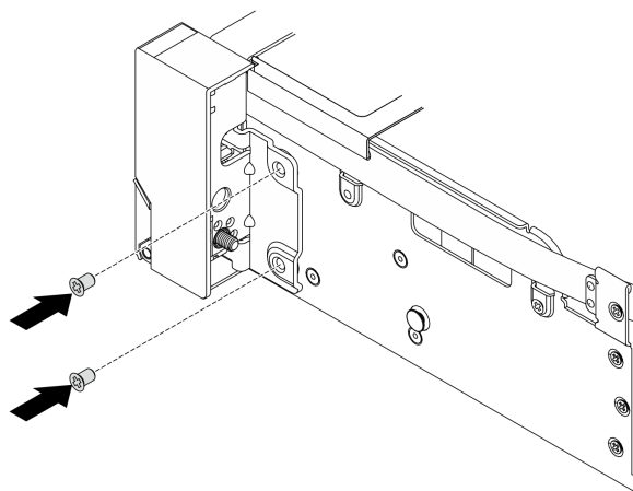
図 224. ねじの取り付け
