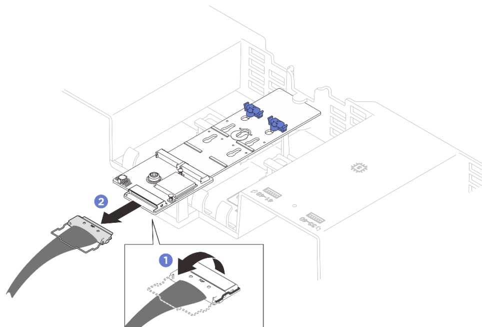
図 34. M.2 ブート・アダプターのケーブルの取り外し
