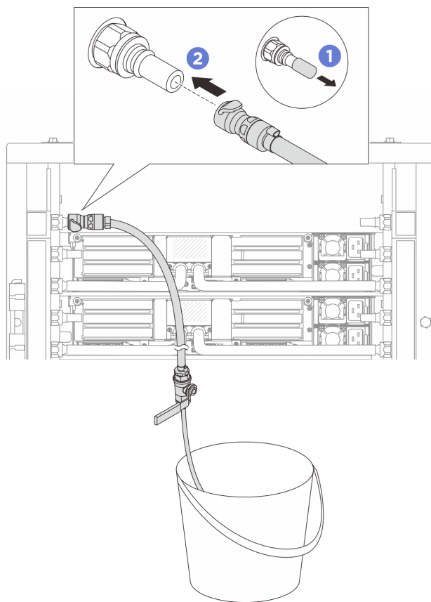
図 163. 供給側へのブリーダー・キットの取り付け
