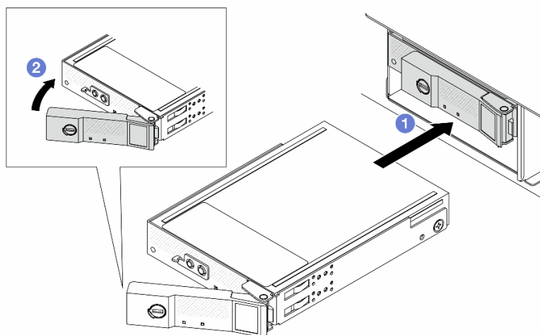
図 48. E3.S CMM の取り付け
