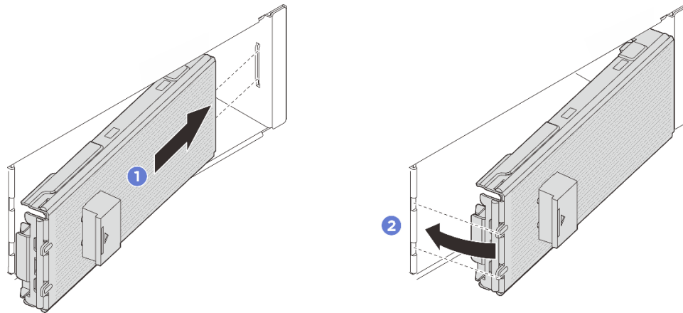
図 63. E3.S ベゼルの取り付け
