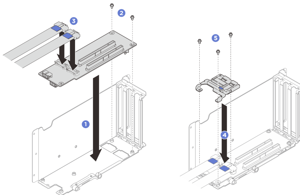
図 197. PCIe ライザー・カードの取り付け
