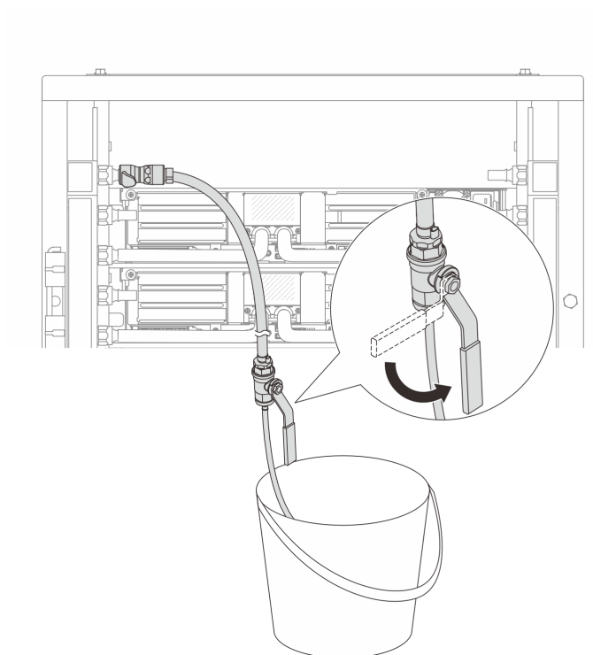
図 165. 供給側のブリーダーのバルブを開く
