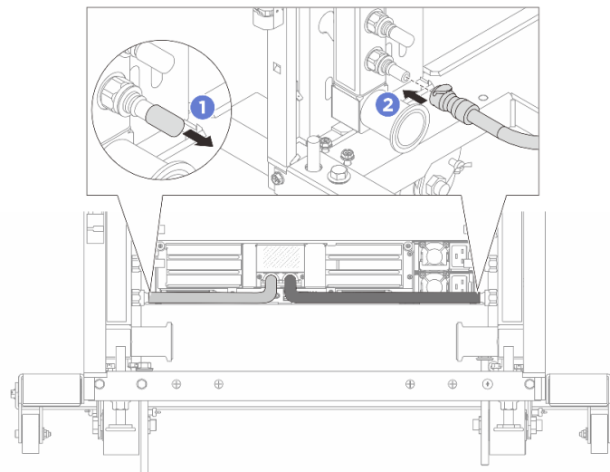
図 145. クイック・コネクト・プラグの取り付け
