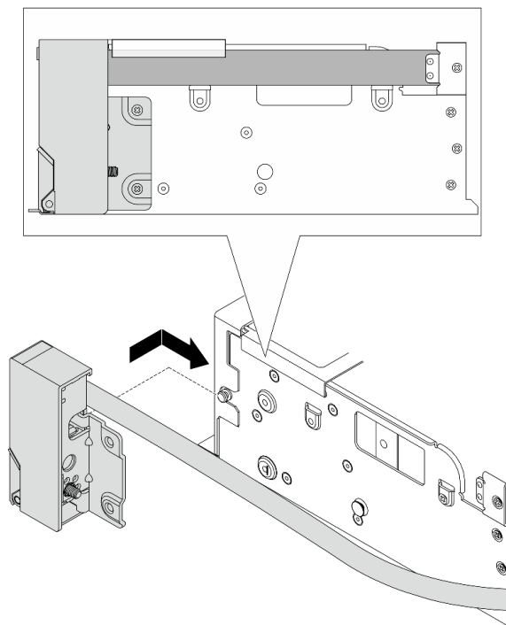
図 223. ラック・ラッチの取り付け
