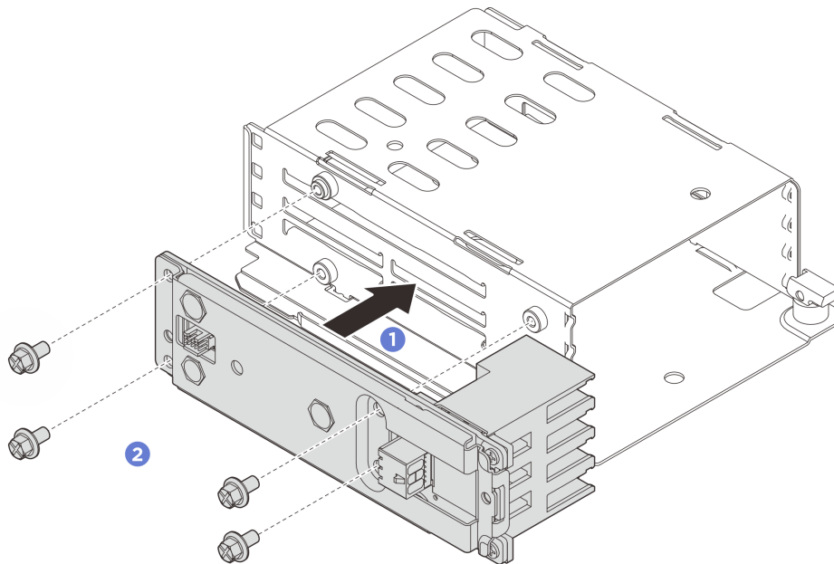
図 66. バックプレーン・アセンブリーの取り付け
