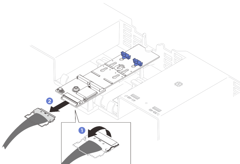
図 28. M.2 ブート・アダプターのケーブルの取り外し
