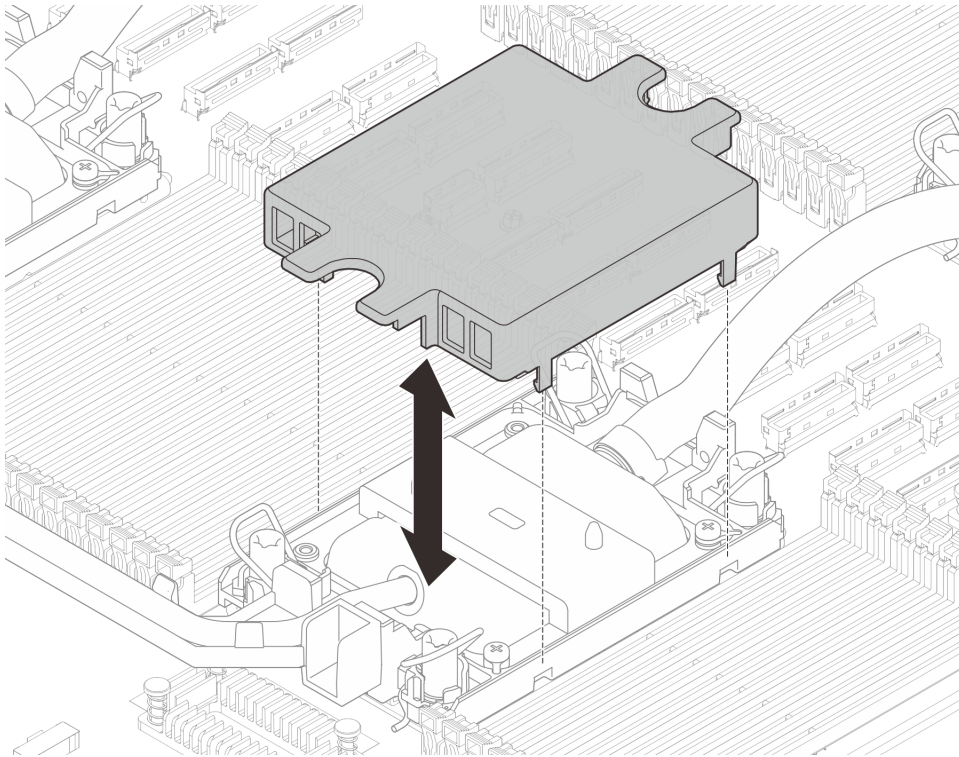
図 276. コールド・プレート・カバーの取り外し
