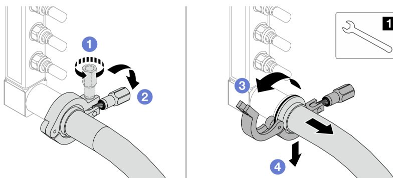
図 159. ホース・キットからの多岐管の分離
