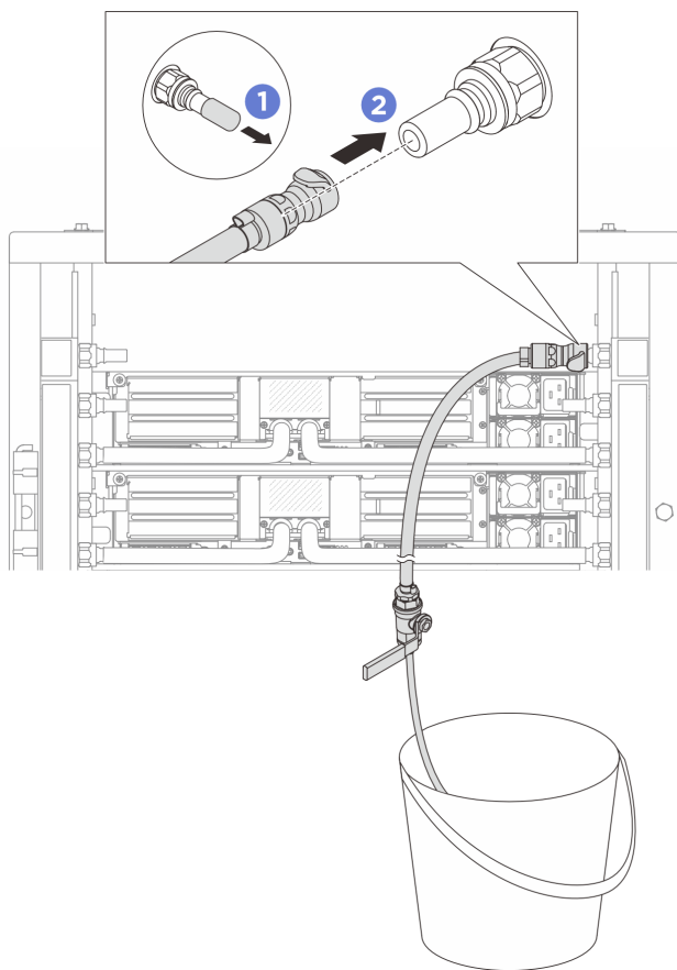
図 166. リターン側へのブリーダー・キットの取り付け
