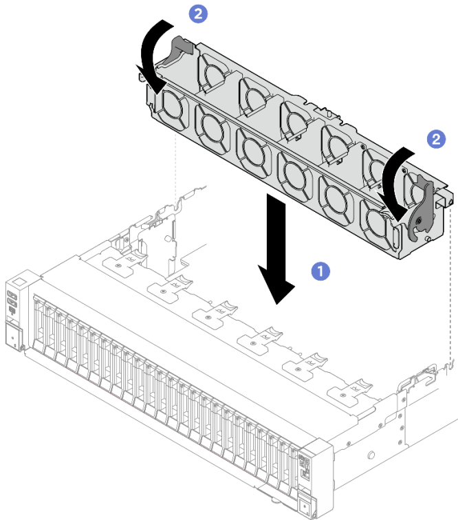
図 70. ファン・ケージの取り付け
