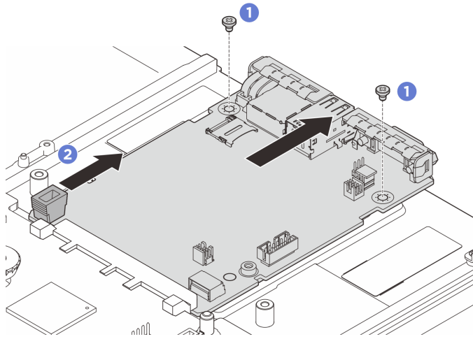
図 244. システム I/O ボードの取り外し
