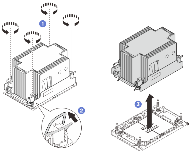
図 210. 2U 標準 PHM の取り外し
