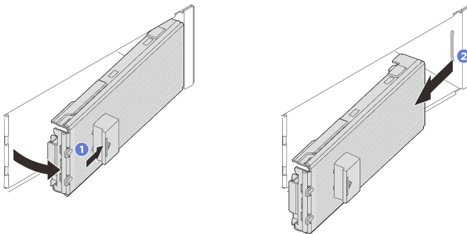
図 43. E3.S ベゼルの取り外し
