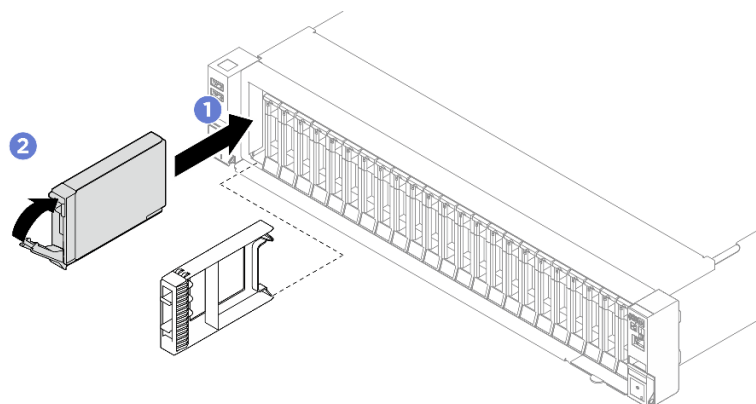
図 26. 2.5 インチ ホット・スワップ・ドライブの取り付け
