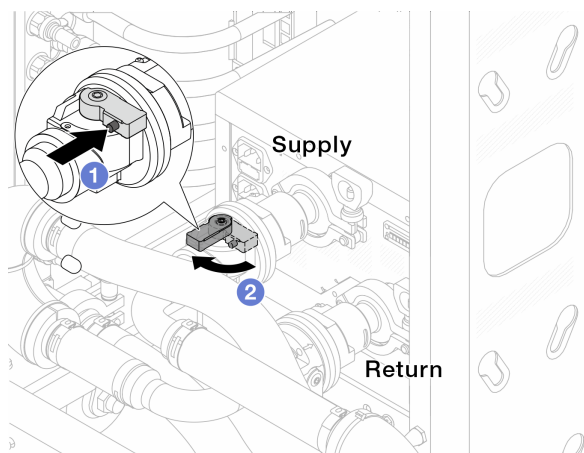
図 147. ボール・バルブを開く
