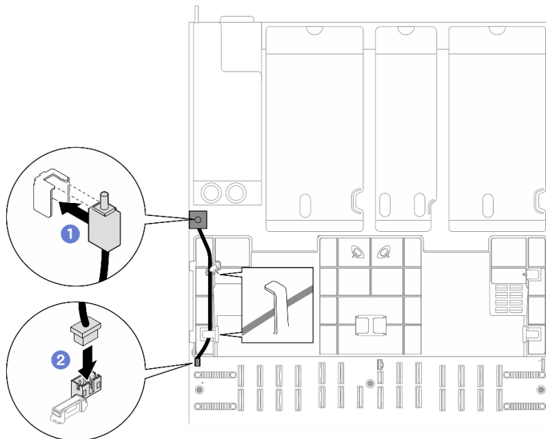
図 95. 侵入検出スイッチの取り付け
