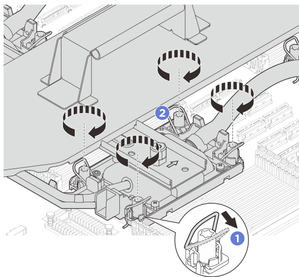
図 109. Torx T30 ナットの締め付け
