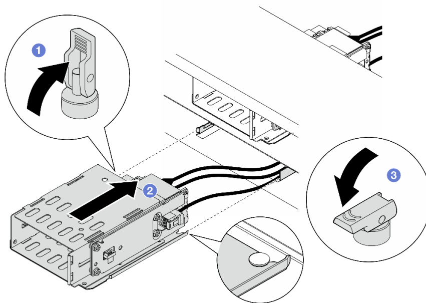
図 55. E3.S 2T ケージの取り付け
