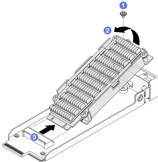
図 84. ヒートシンク付き M.2 ドライブを取り外す
