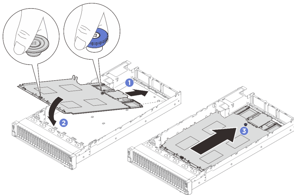
図 250. システム・ボード・アセンブリーの取り付け
