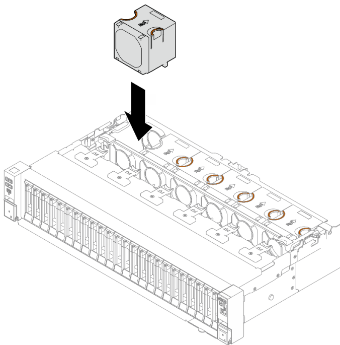
図 71. ファンの取り付け
