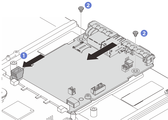
図 249. システム I/O ボードの取り付け
