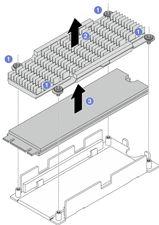
図 86. M.2 ドライブとヒートシンクの分離
