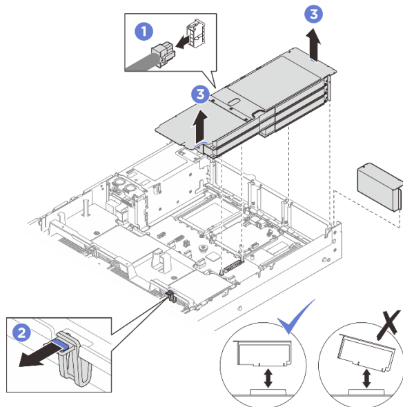
図 184. PCIe FHFL ライザーの取り外し
