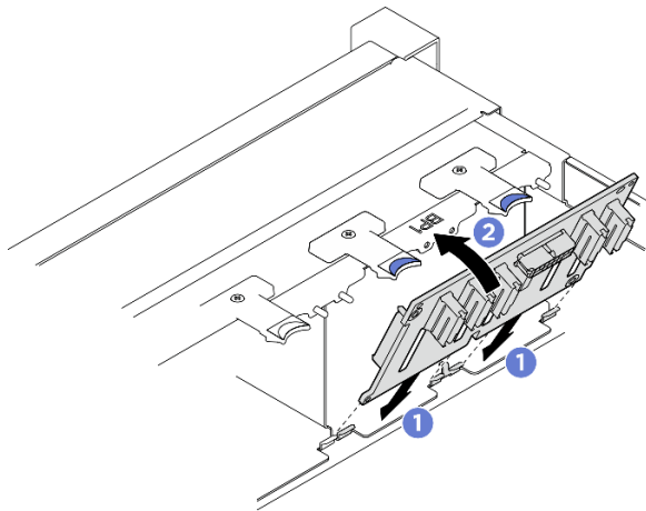
図 25. 2.5 インチ ドライブ・バックプレーンの取り付け
