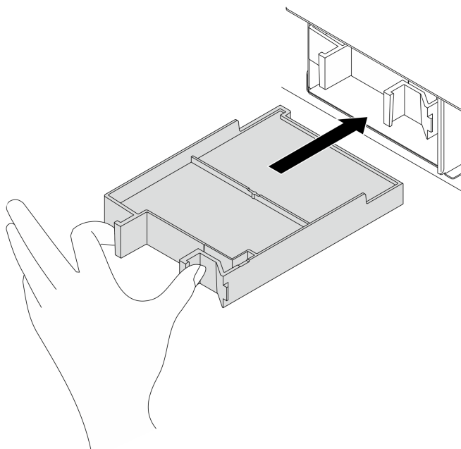
図 49. CMM ベイ・フィラーの取り付け
