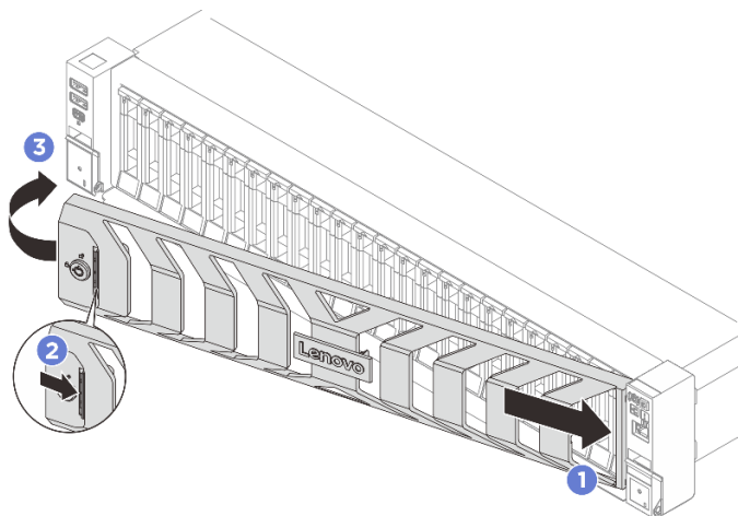
図 235. セキュリティー・ベゼルの取り付け
