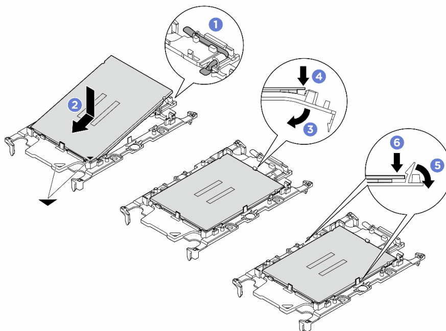
図 104. プロセッサ・キャリアの取り付け
