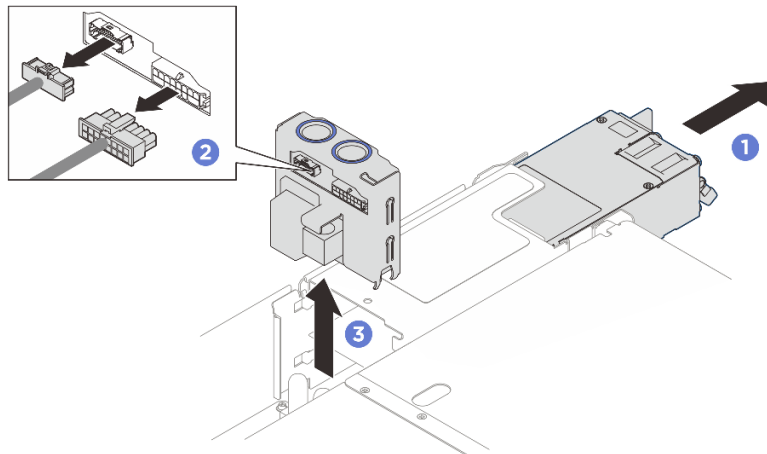
図 204. 分電盤の取り外し
