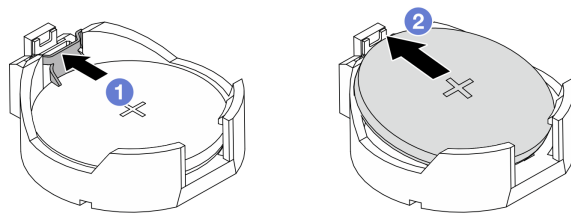
図 40. CMOS バッテリーの取り外し
