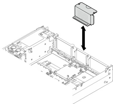
図113. ライザー・フィラーの取り付け
