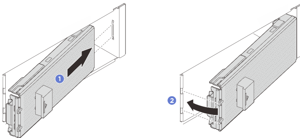
図 51. E3.S ベゼルの取り付け
