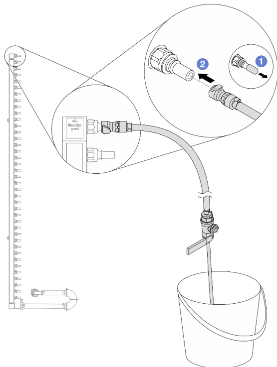
図 133. 供給側へのブリーダー・キットの取り付け
