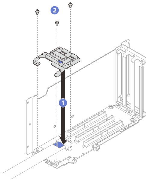
図 201. PCIe 保持具の取り付け
