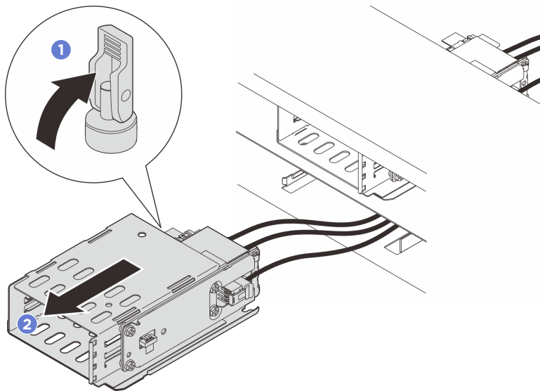
図 64. E3.S 1T ケージの取り外し
