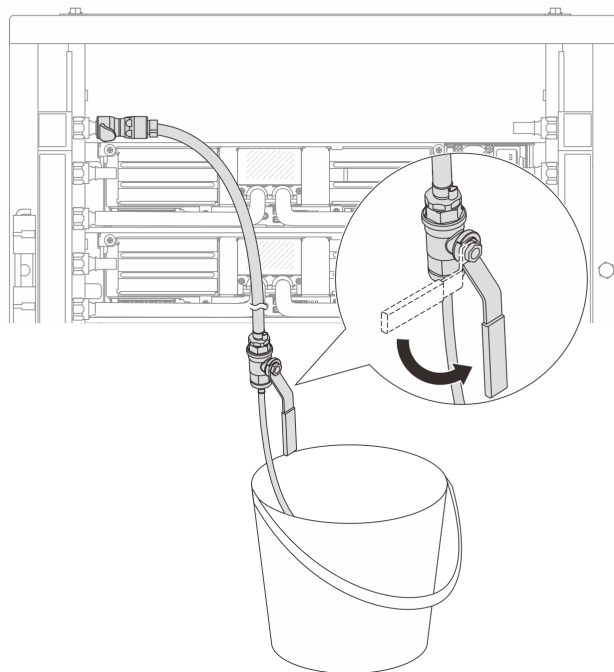
図 169. 供給側のブリーダーのバルブを開く
