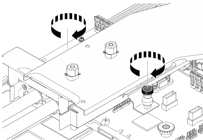
図 108. コールド・プレート・アセンブリーの取り付け
