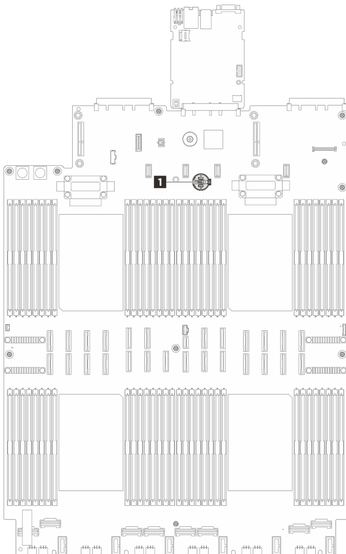
図 41. CMOS バッテリー・ソケットの位置
