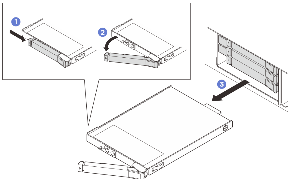
図 57. E3.S ホット・スワップ・ドライブの取り外し
