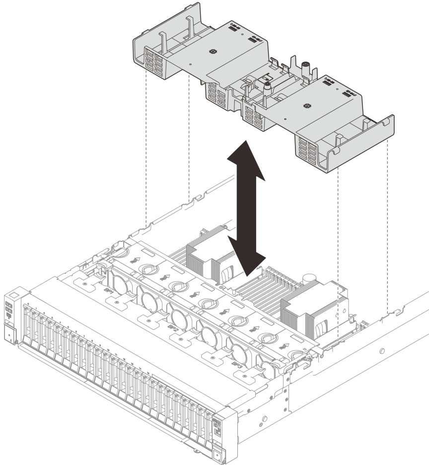
図 30. 前面エアー・バッフルの取り付け
