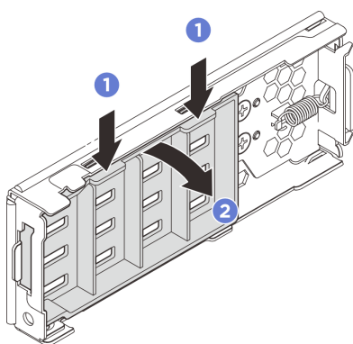
図 50. 内板の取り外し
