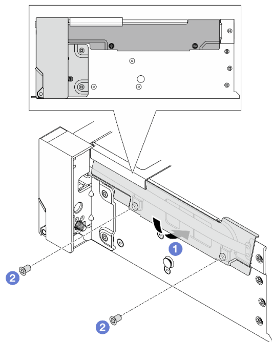
図 225. ケーブル保持具の取り付け
