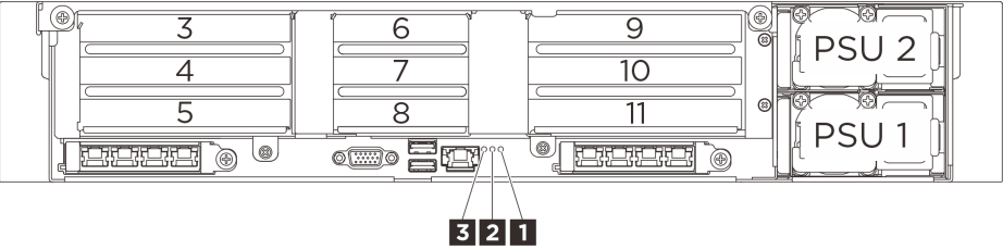
図 271. 背面システム LED
