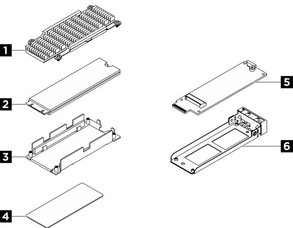
図 81. ホット・スワップ M.2 ドライブ・アセンブリーの部品
