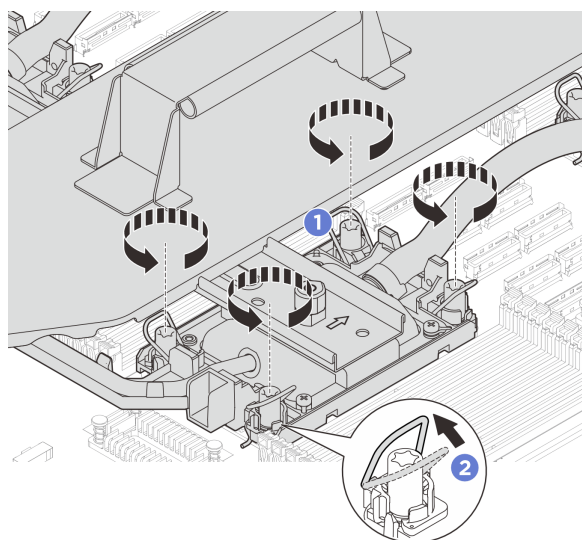
図 101. Torx T30 ナットを緩める
