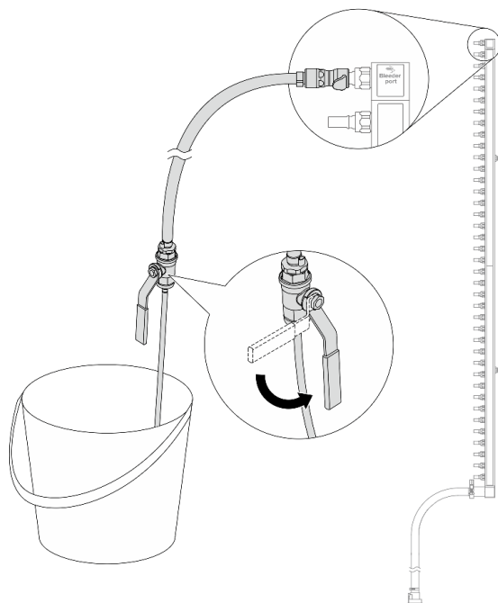
図 158. ブリーダー・バルブを開く
