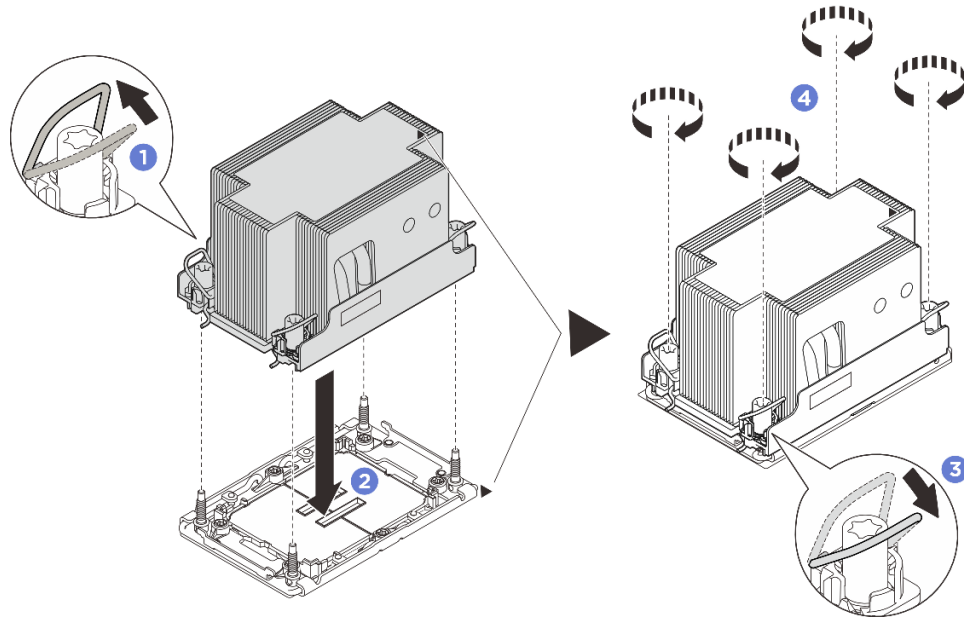
図 218. 2U 標準 PHM の取り付け
