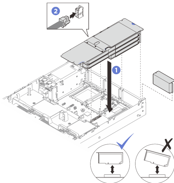
図 192. PCIe FHFL ライザーの取り付け
