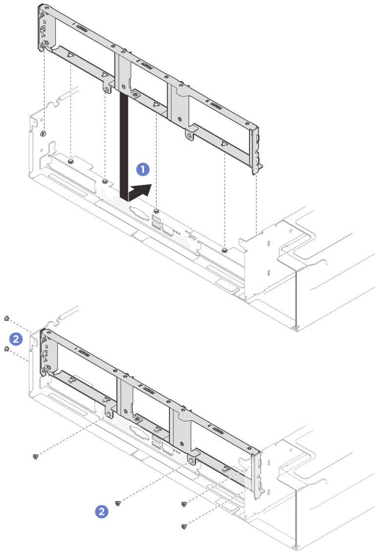
図 231. 背面の壁の取り付け
