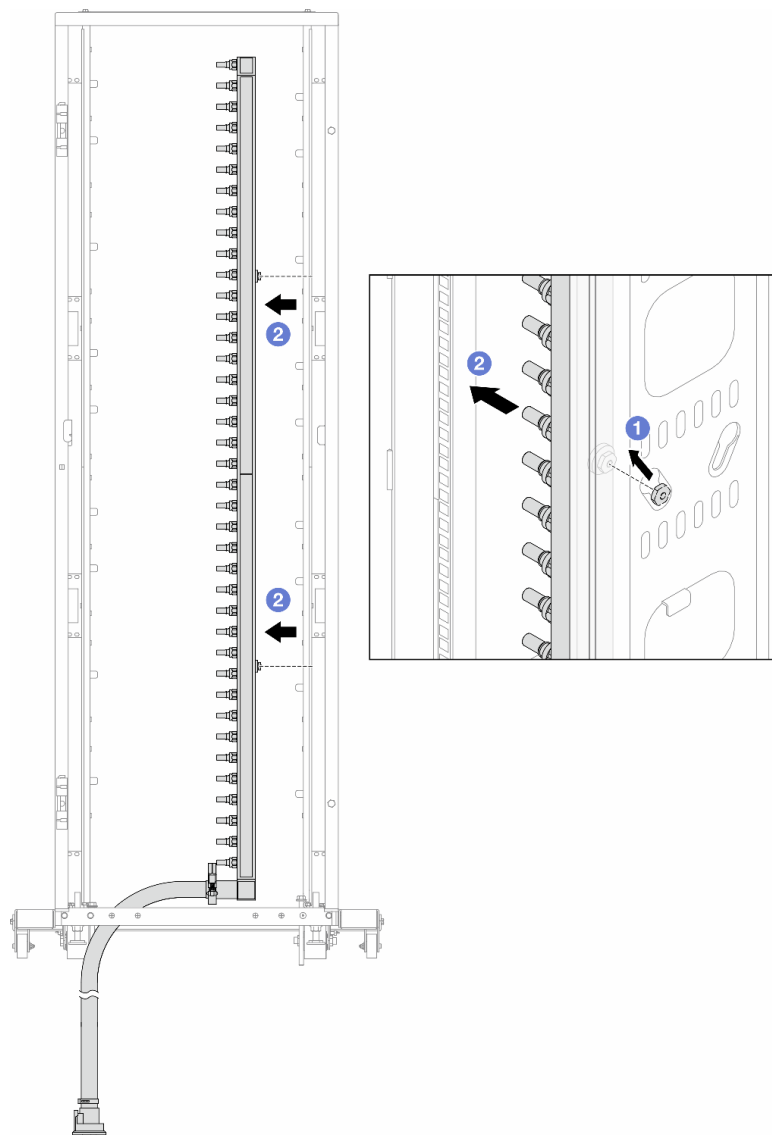
図 154. 多岐管の取り外し
