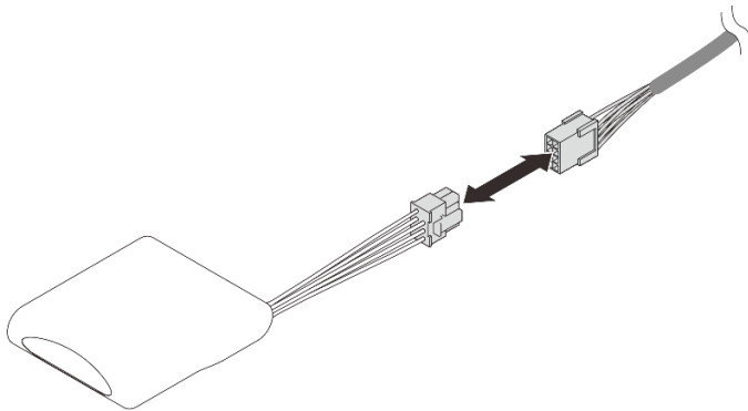
図 27. フラッシュ電源モジュール・ケーブルの切り離し
