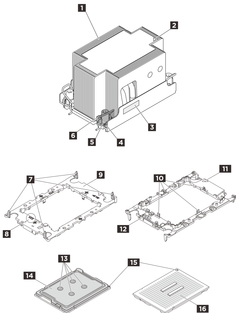
図 214. PHM コンポーネント
