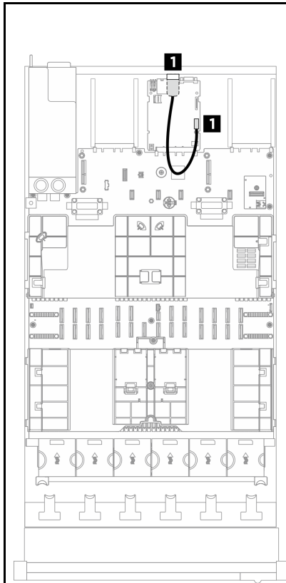
図 240. 3 個の PCIe ライザーを搭載したサーバー・モデルのシリアル・ポート・モジュールのケーブル配線
