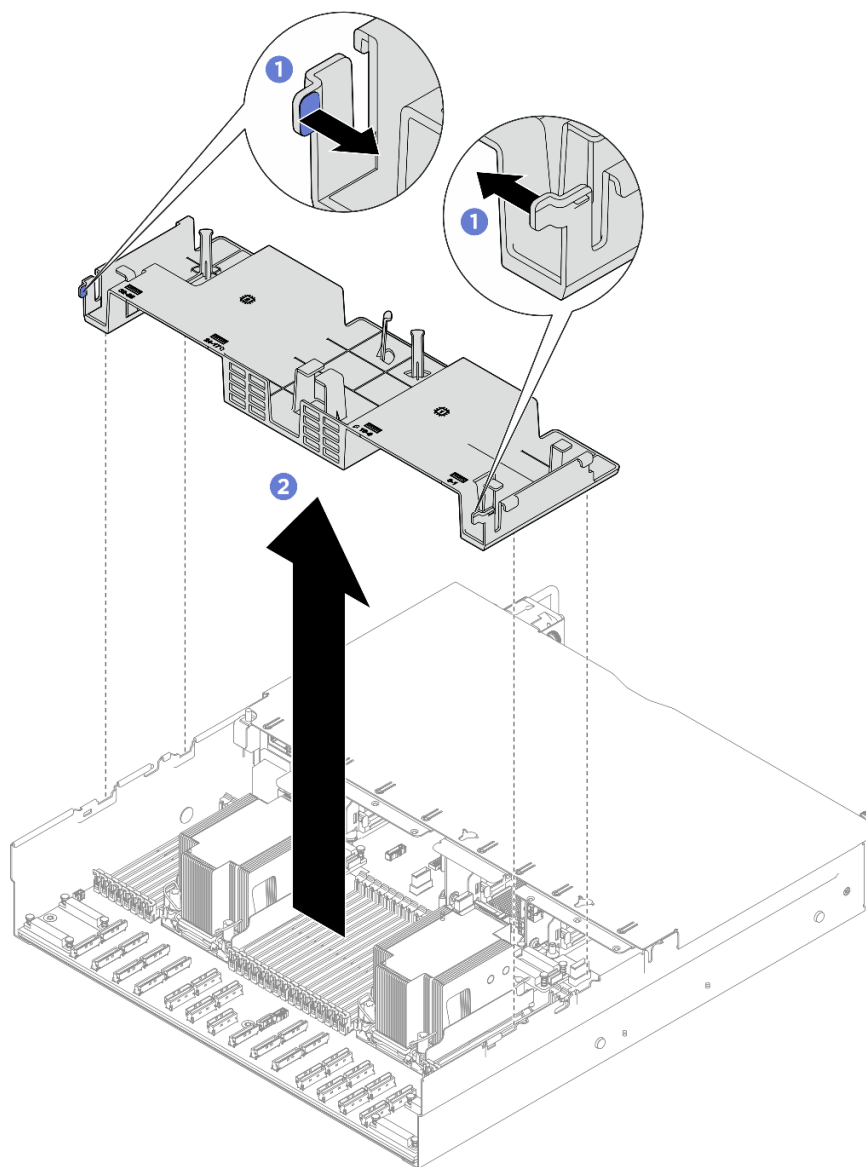
図 35. 背面エアー・バッフルの取り外し
