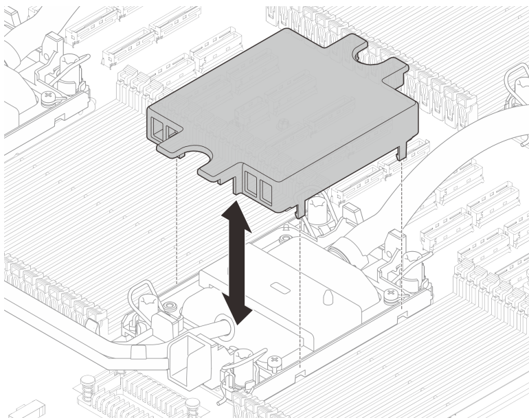
図 98. コールド・プレート・カバーの取り外し
