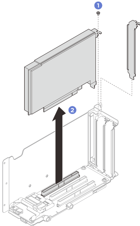
図 185. PCIe アダプターの取り外し
