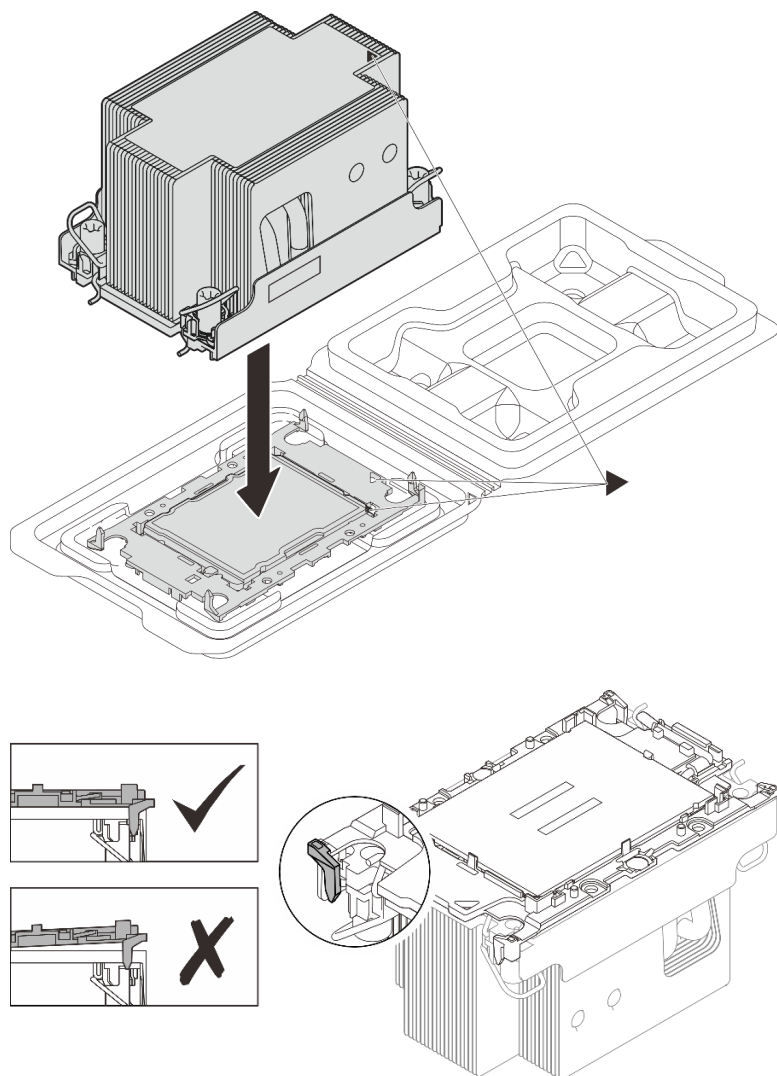
図 217. 配送用トレイのプロセッサーで PHM を取り付けます。
