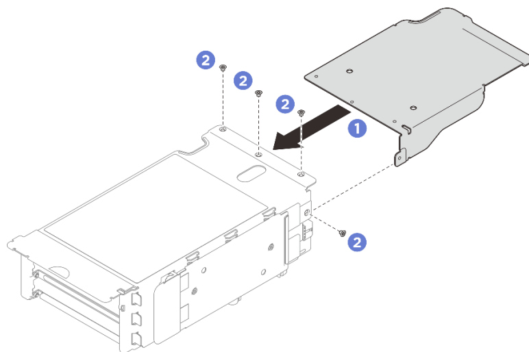
図 203. PCIe ライザー・エクステンダーの取り付け
