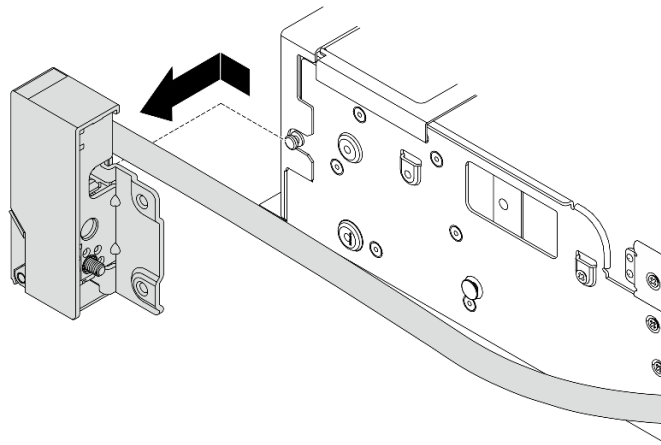
図 222. ラック・ラッチの取り外し
