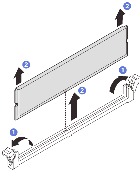
図 172. メモリー・モジュールの取り外し
