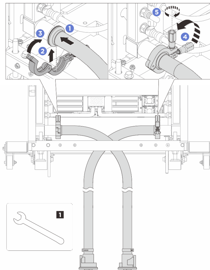
図 162. ホース・キットの取り付け
