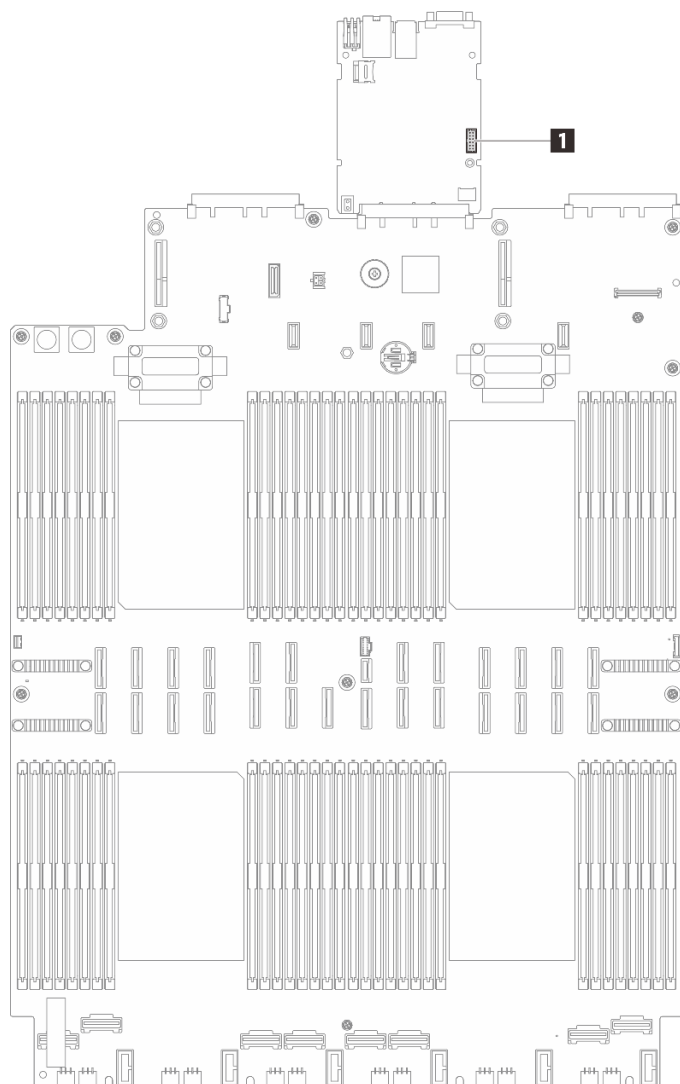
図 239. シリアル・ポート・コネクタの位置
