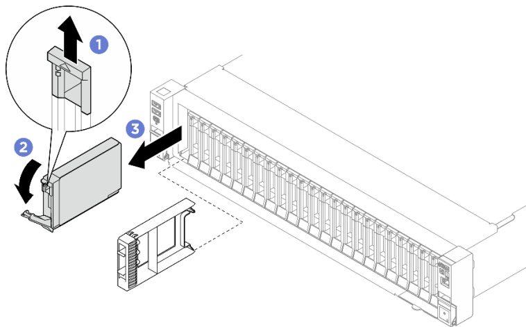
図 23. 2.5 インチ ホット・スワップ・ドライブの取り外し
