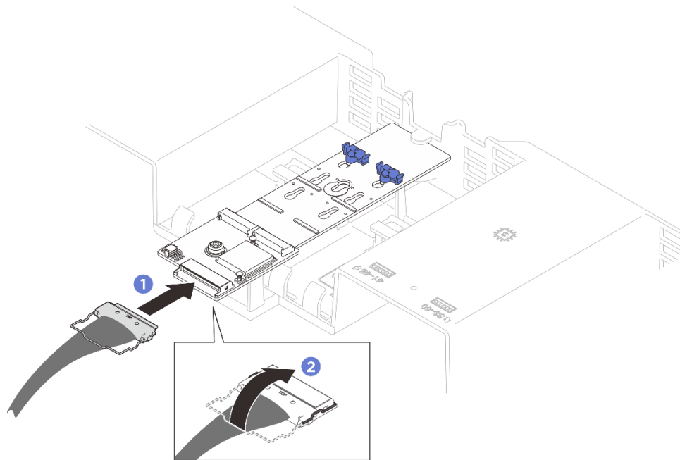
図 119. M.2 ブート・アダプターのケーブル接続
