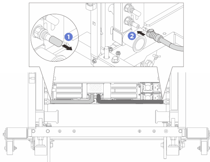
図 161. クイック・コネクト・プラグの取り付け
