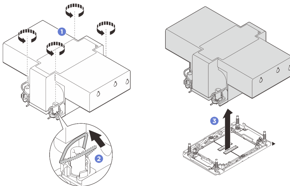
図 211. 2U パフォーマンス PHM の取り外し
