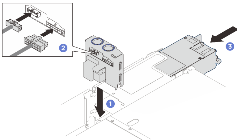
図 206. 分電盤の取り付け
