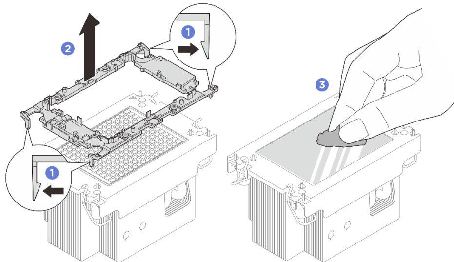
図213. ヒートシンクからプロセッサ・キャリアを取り外す
