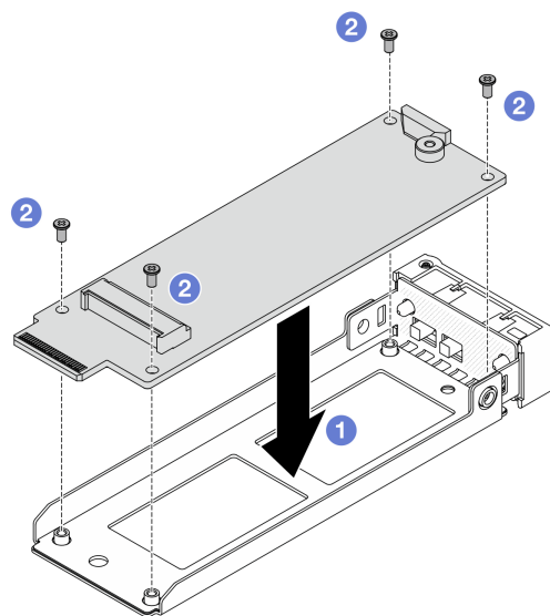
図 90. M.2 変換コネクタの取り付け
