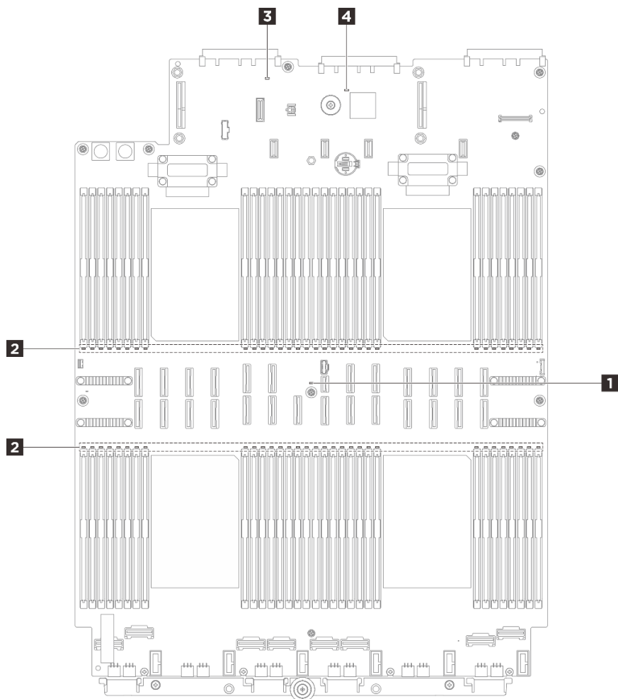
図 272. プロセッサ・ボード LED
