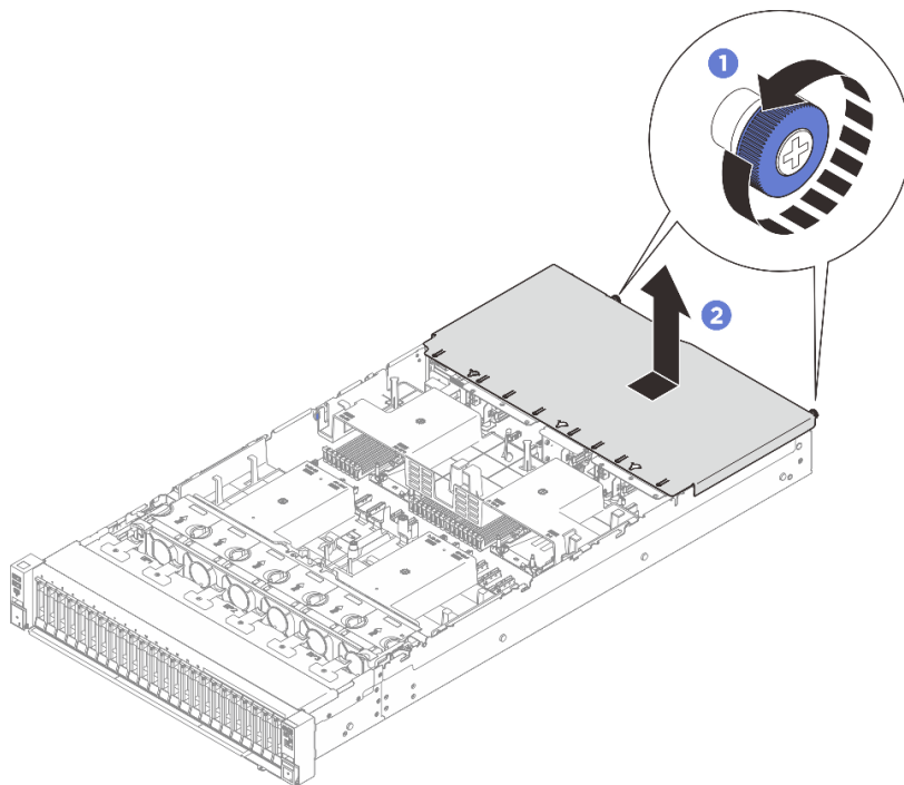
図 253. 背面トップ・カバーの取り外し
