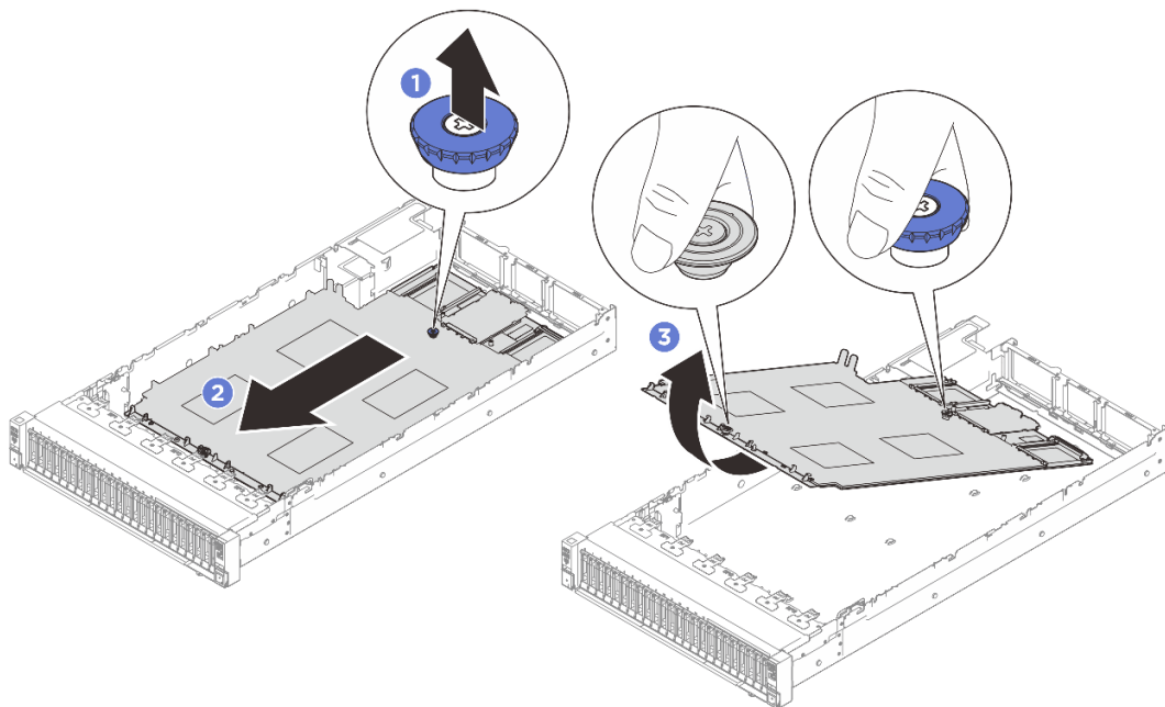
図 243. システム・ボード・アセンブリーの取り外し
