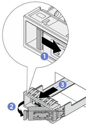
図 92. M.2 ドライブ・トレイの取り外し
