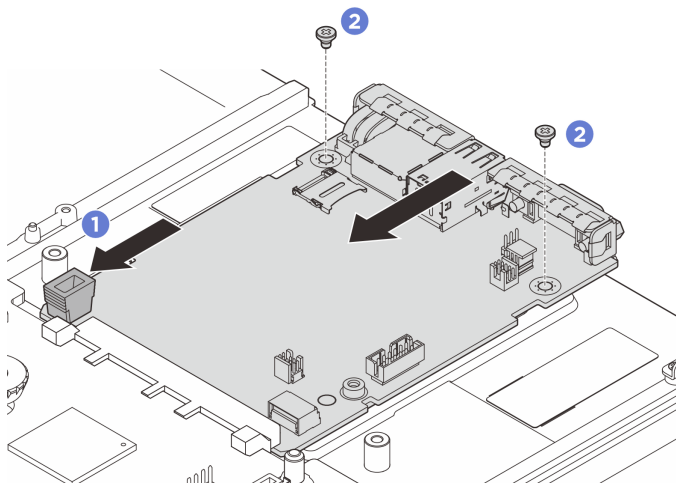
図 245. システム I/O ボードの取り付け
