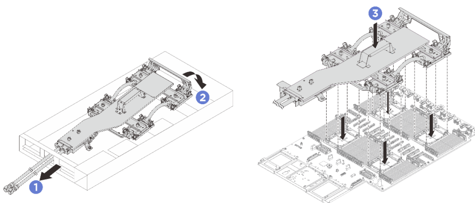
図 107. コールド・プレート・アセンブリーの取り付け
