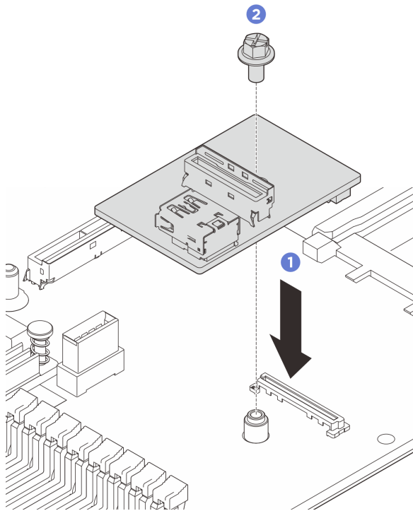
図 258. USB I/O ボードの取り付け
