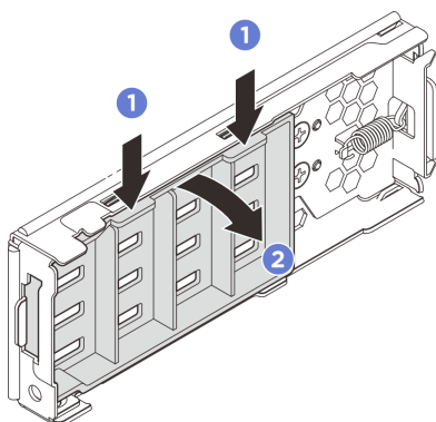
図 62. 内板の取り外し
