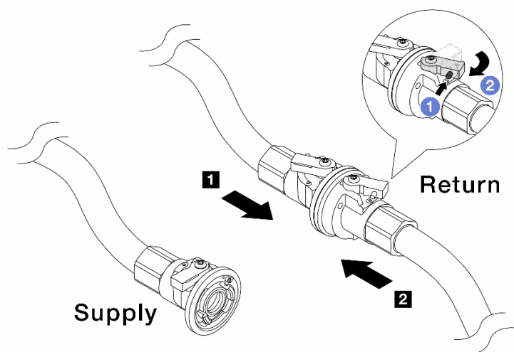
図 164. ファシリティー供給から多岐管のリターンへ
