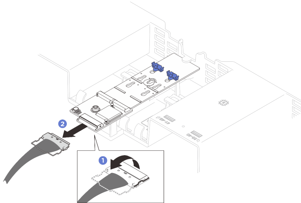
図 116. M.2 ブート・アダプターのケーブルの取り外し
