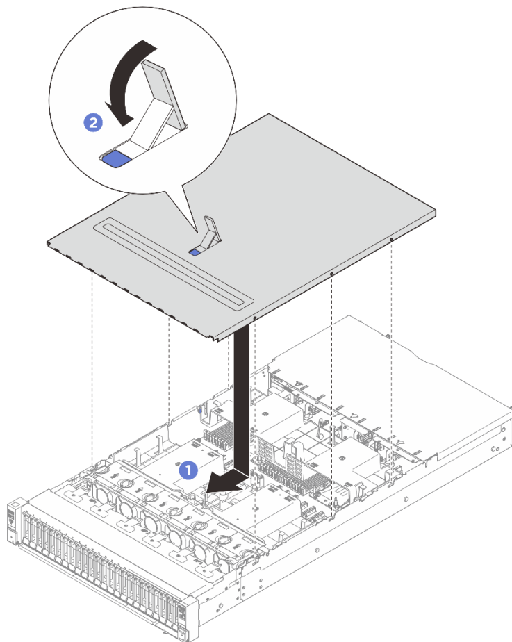
図 255. 前面トップ・カバーの取り付け
