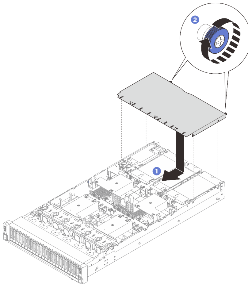
図 254. 背面トップ・カバーの取り付け
