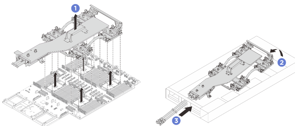
図 103. コールド・プレート・アセンブリの取り外し
