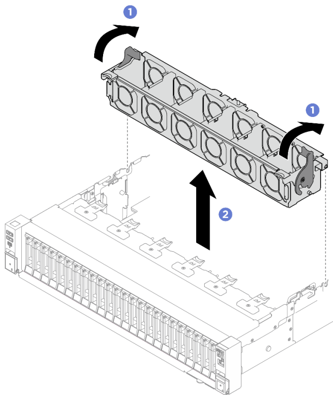
図 69. ファン・ケージの取り外し
