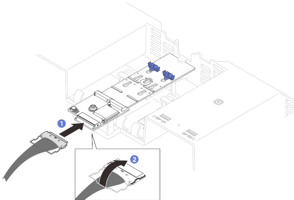
図 31. M.2 ブート・アダプターのケーブル接続
