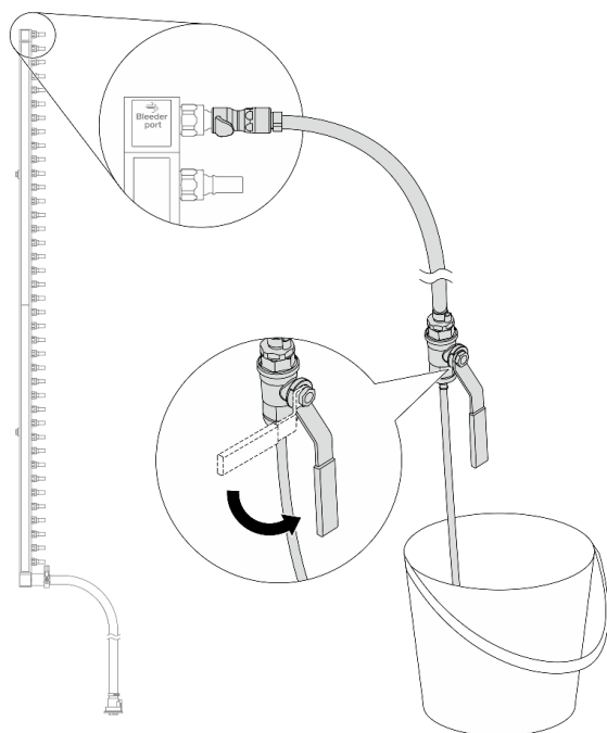
図 156. ブリーダー・バルブを開く
