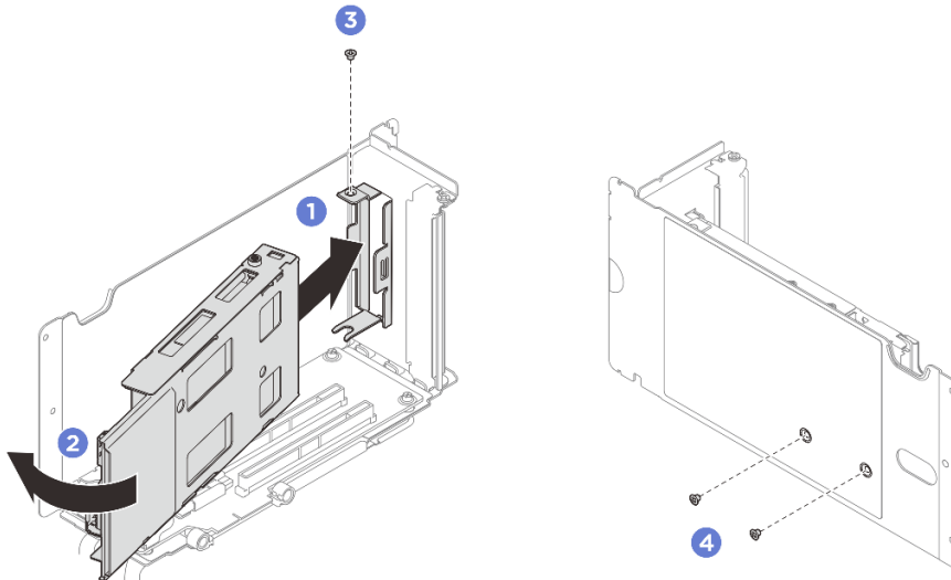
図 229. M.2 ドライブ・ケージの取り付け
