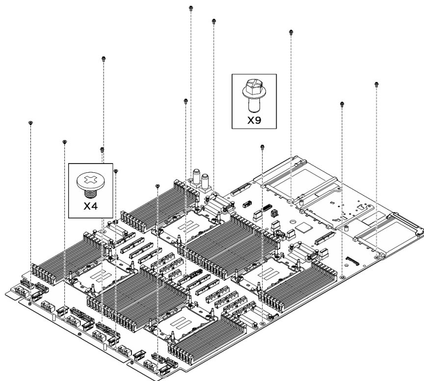
図 279. ねじの取り外し
