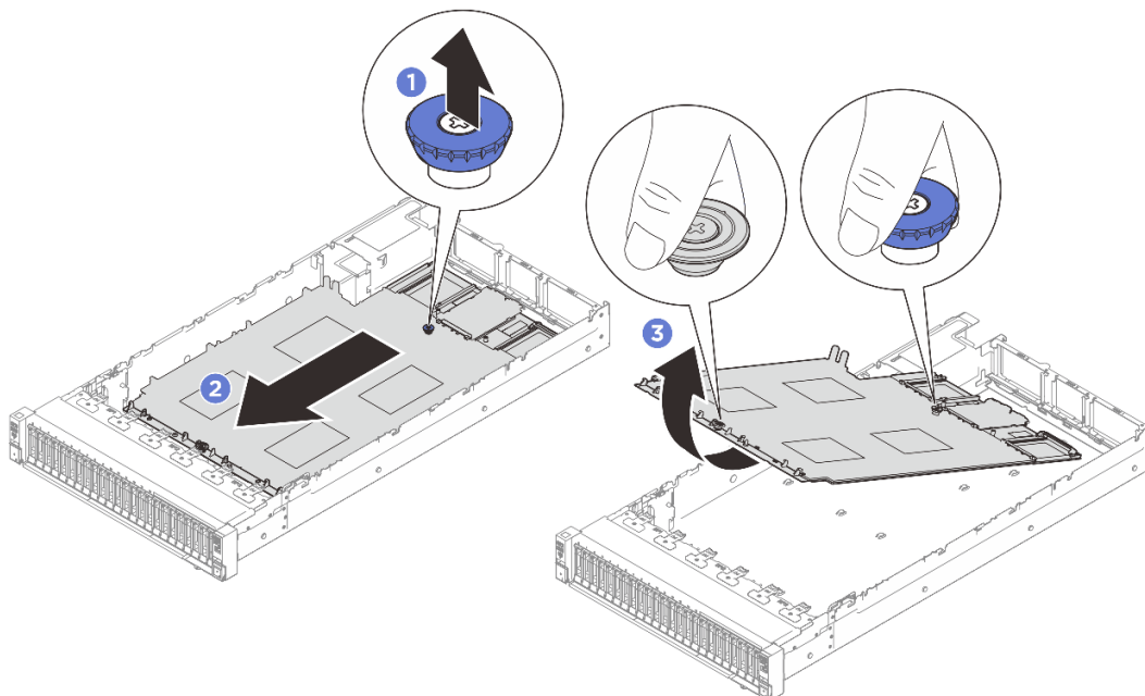
図 247. システム・ボード・アセンブリーの取り外し
