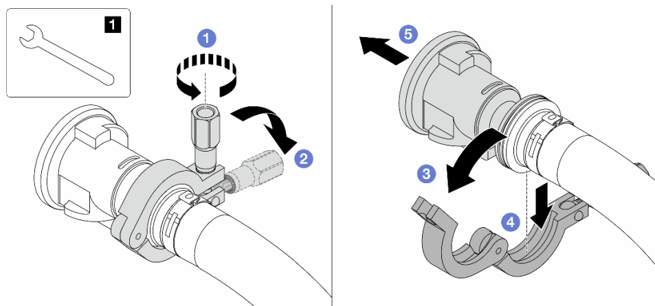
図 139. ボール・バルブの取り外し
