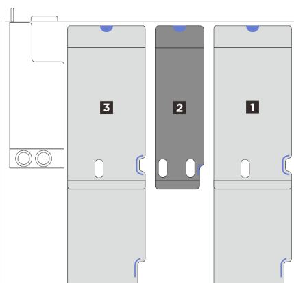
図 180. 3 個の PCIe ライザーおよびライザー・エクステンダーを搭載したサーバー・モデル
