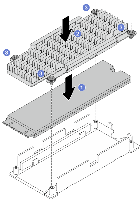
図 89. ヒートシンクと M.2 ドライブの組み立て
