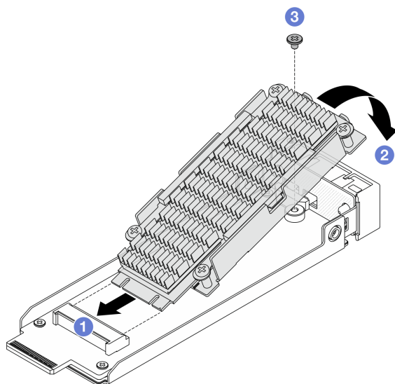
図 91. ヒートシンクが付いた M.2 ドライブの取り付け
