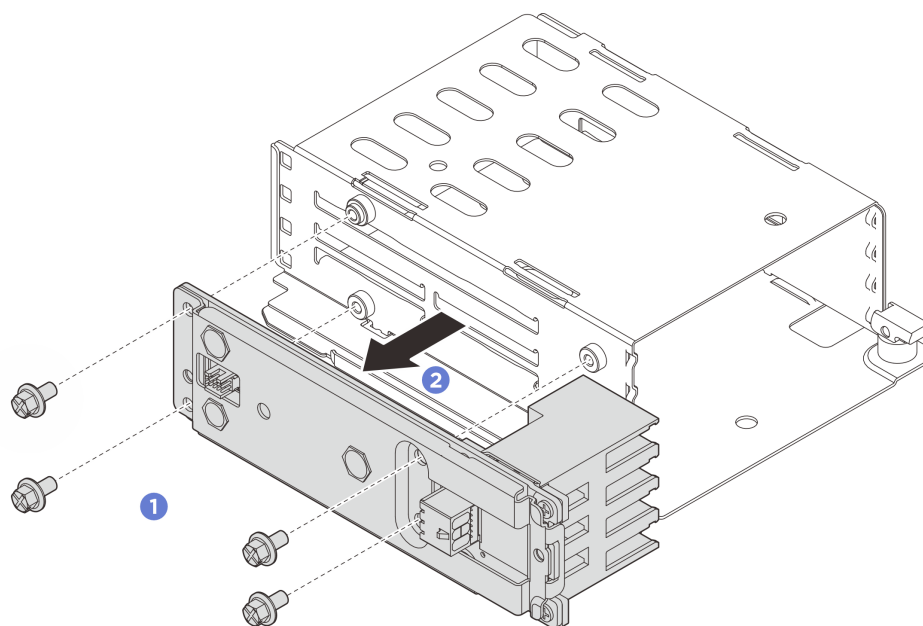
図 65. バックプレーン・アセンブリーの取り外し
