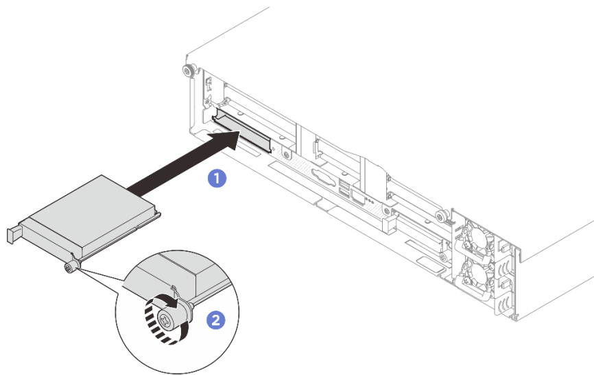
図 178. OCP モジュールの取り付け
