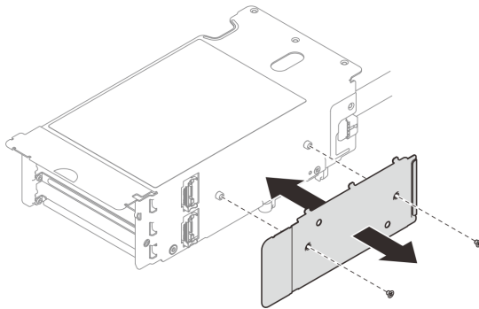
図 196. ケーブル・カバーの取り外し
