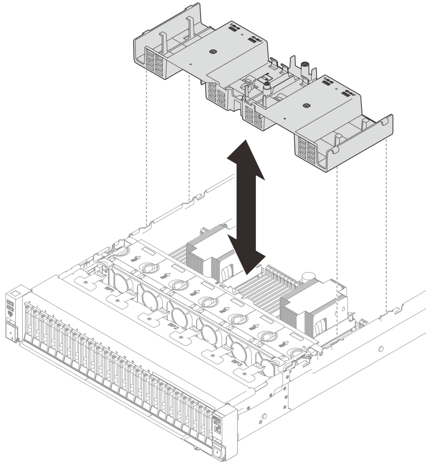
図 29. 前面エアー・バッフルの取り外し
