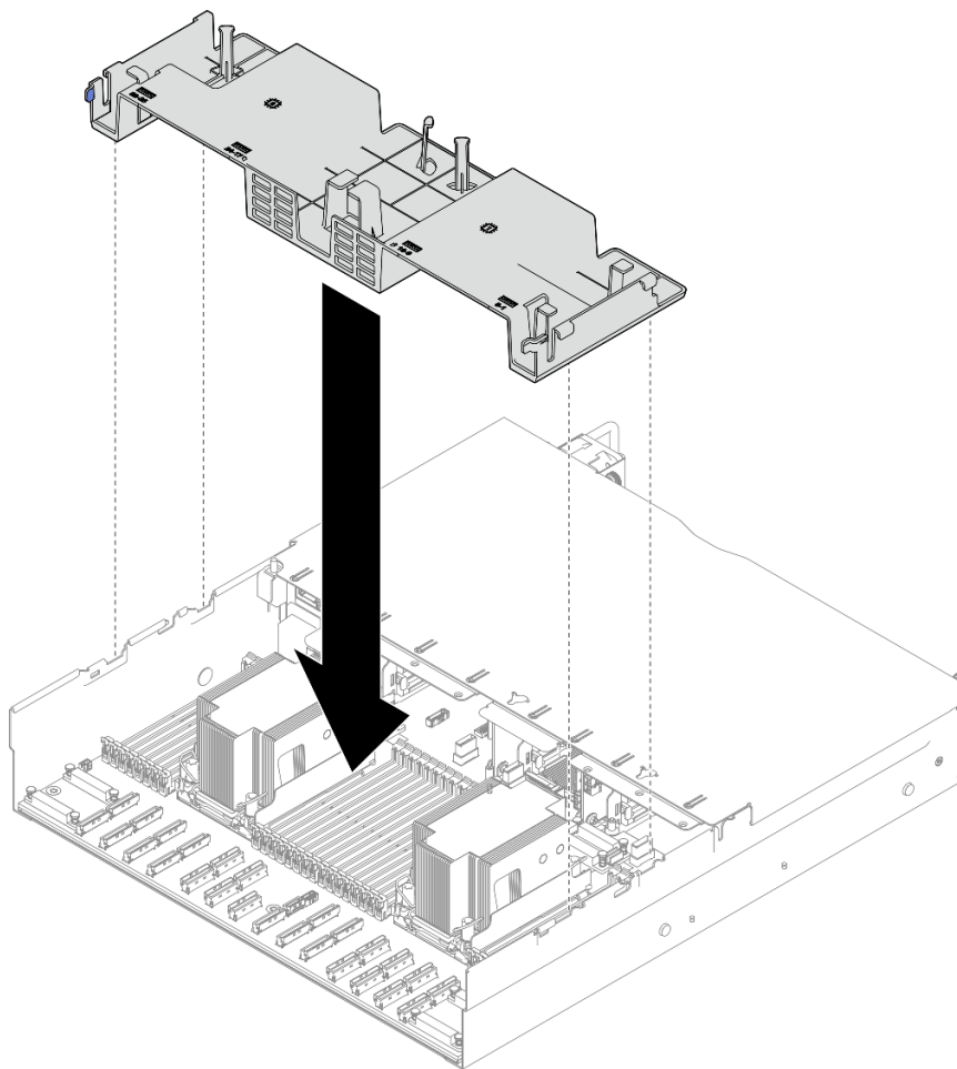
図 36. 背面エアー・バッフルの取り付け
