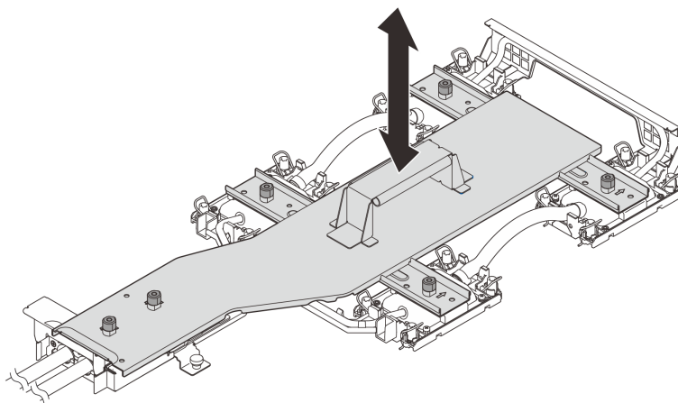
図 99. コールド・プレート・キャリアの取り付け
