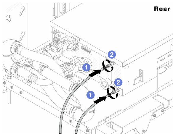
図 144. CDU の背面
