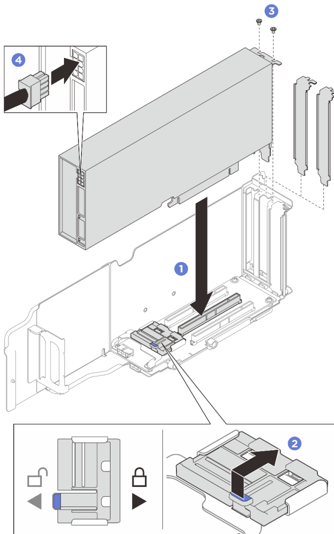
図 80. ダブル・ワイド GPU アダプターの取り付け
