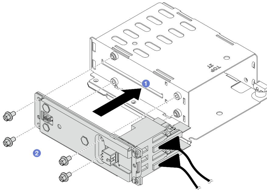
図 54. バックプレーンの取り付け
