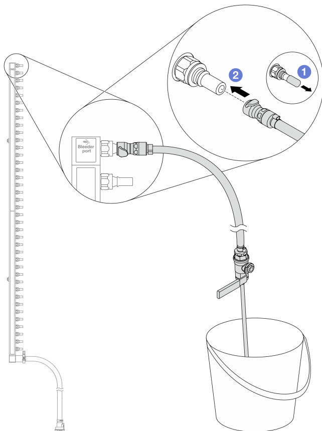
図 155. 供給側へのブリーダー・キットの取り付け
