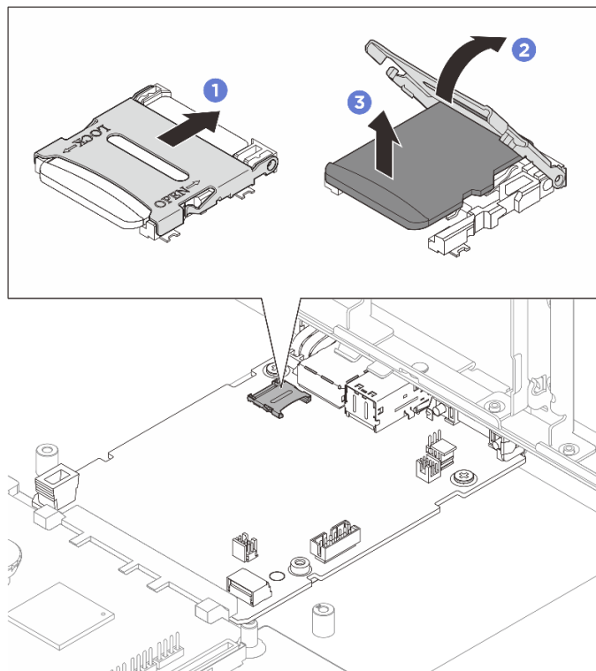
図 175. microSD カードの取り外し
