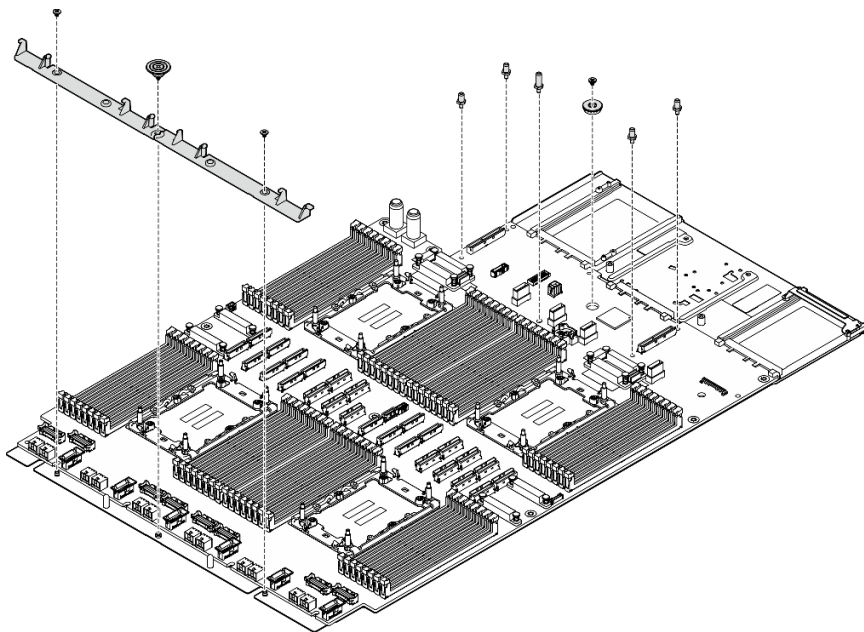
図 278. コンポーネントの取り外し
