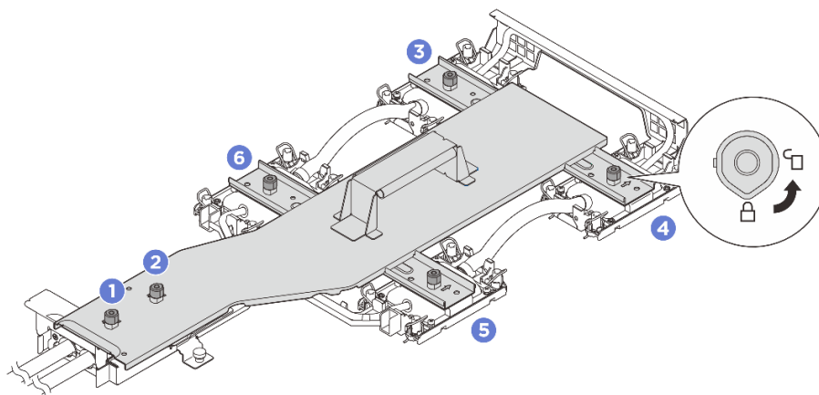
図 110. コールド・プレート・キャリアを緩める
