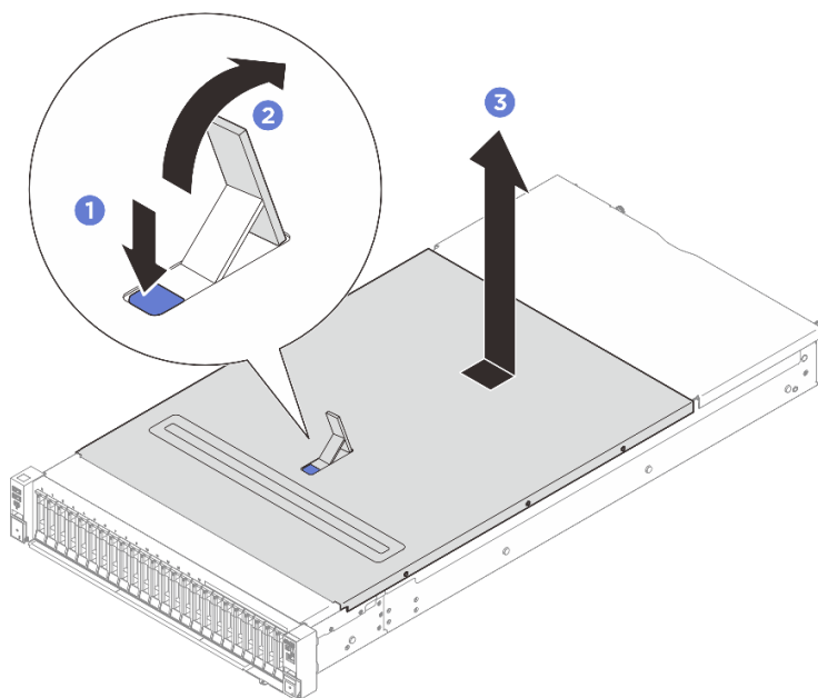
図 252. 前面トップ・カバーの取り外し
