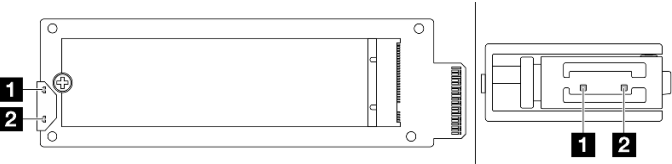
図 269. 背面 M.2 変換コネクタ LED
