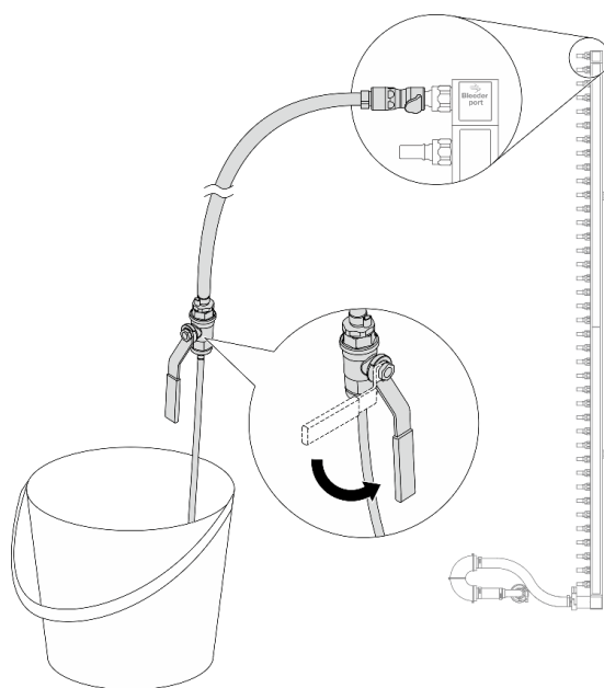
図 136. ブリーダー・バルブを開く
