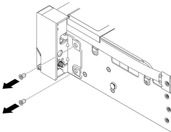
図 221. ねじの取り外し
