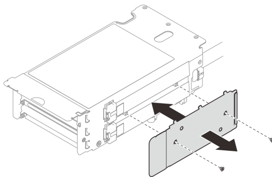
図 193. ケーブル・カバーの取り外し
