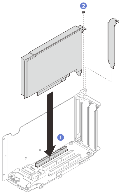
図 186. PCIe アダプターの取り付け
