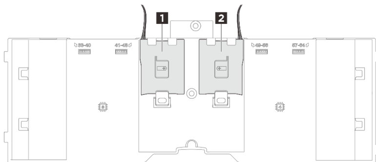
図 74. フラッシュ電源モジュール・スロットの位置
