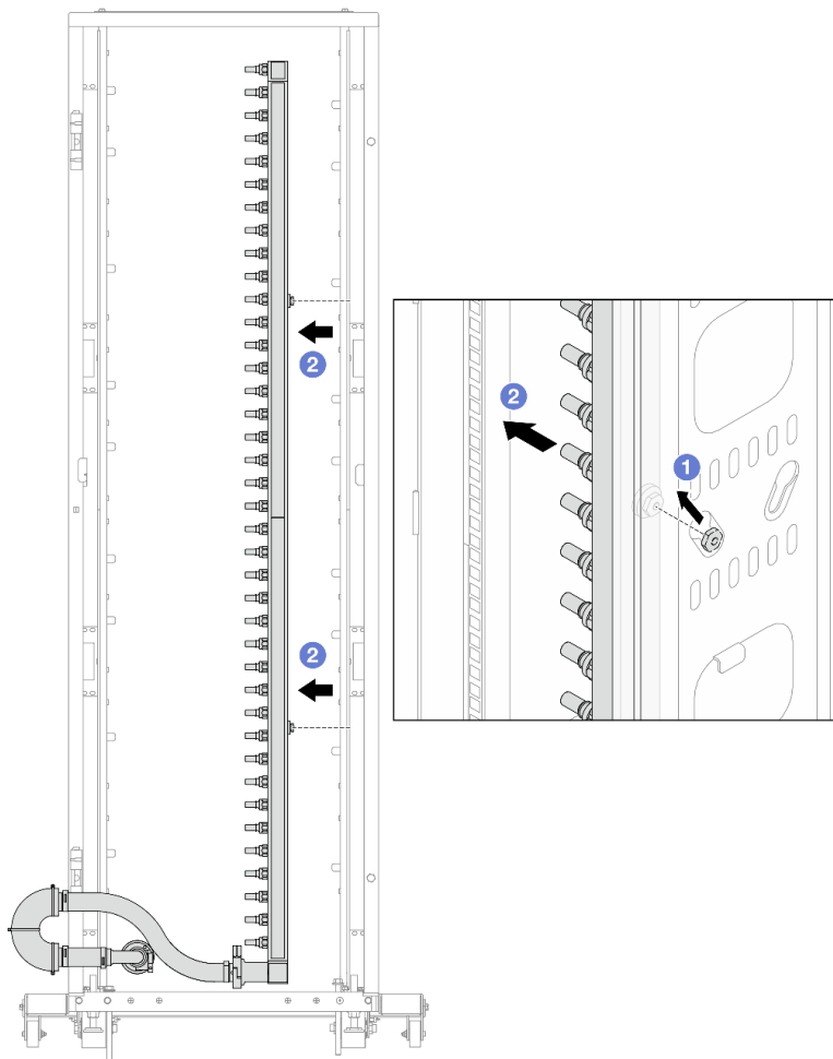
図 132. 多岐管の取り外し
