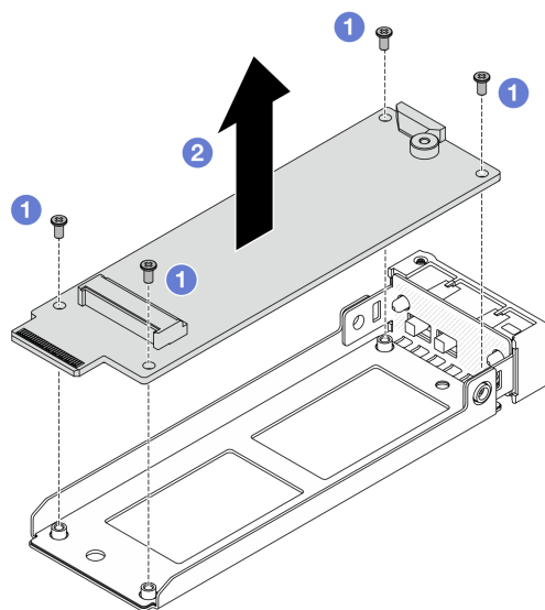
図 85. M.2 変換コネクタの取り外し
