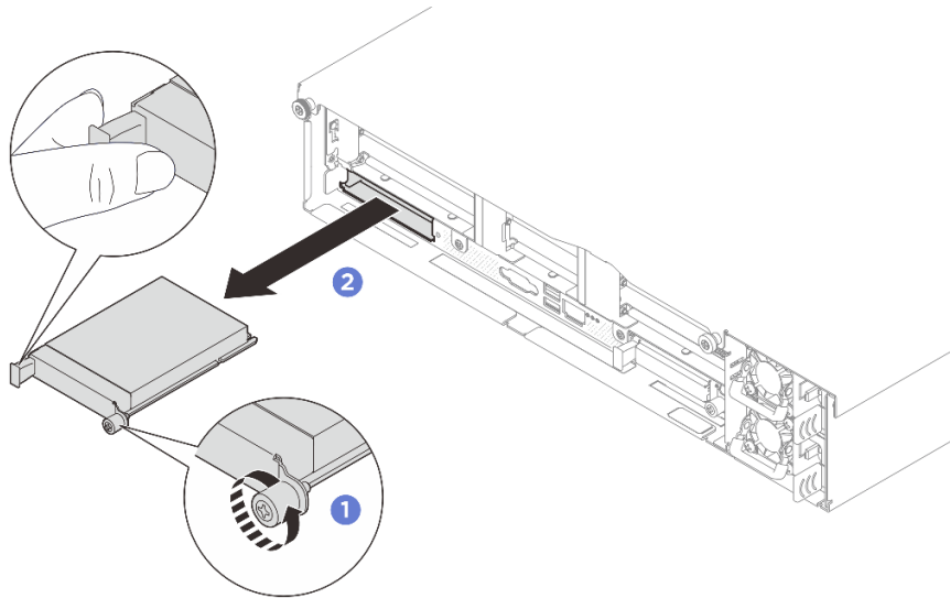
図 177. OCP モジュールの取り外し
