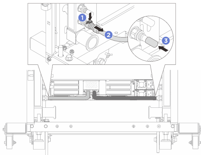
図 130. クイック・コネクト・プラグの取り外し
