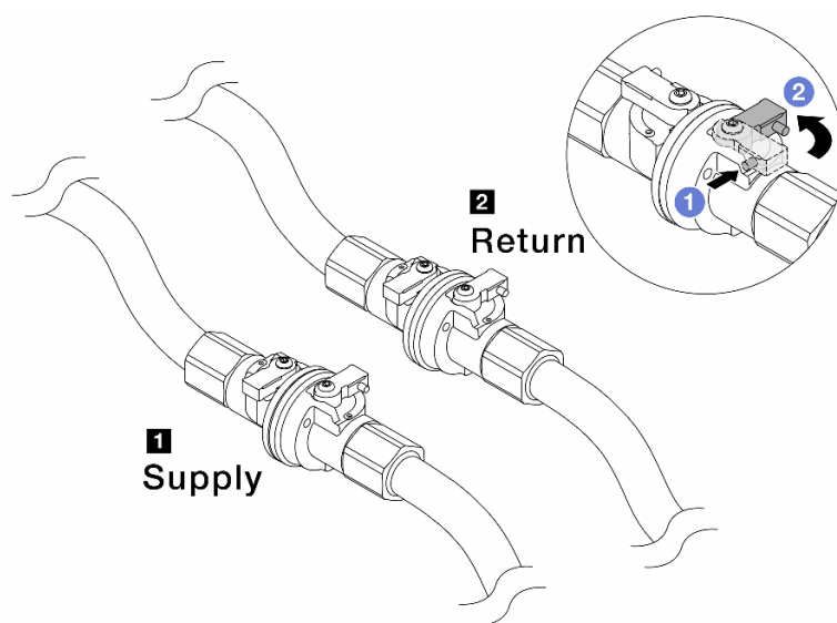
図 152. ボール・バルブを閉じる
