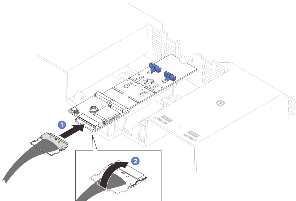
図 37. M.2 ブート・アダプターのケーブル接続
