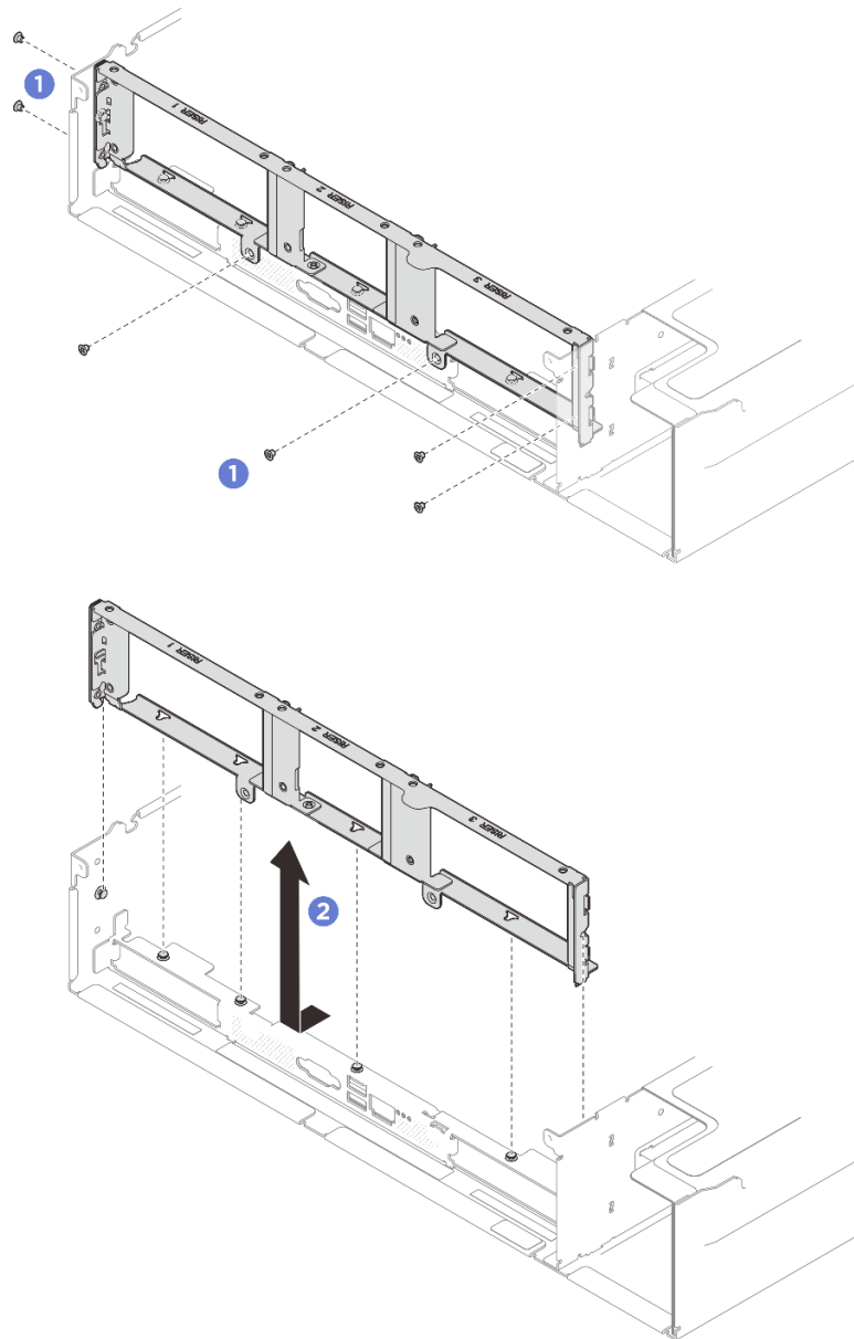
図 230. 背面壁の取り外し
