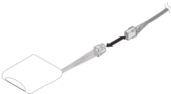
図 33. フラッシュ電源モジュール・ケーブルの切り離し
