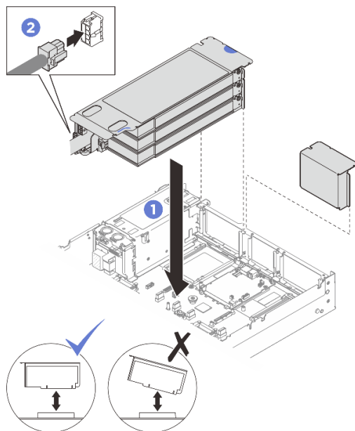
図 190. PCIe LP ライザーの取り付け (電源コネクタあり)
