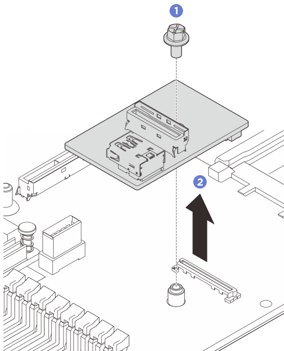
図 257. USB I/O ボードの取り外し
