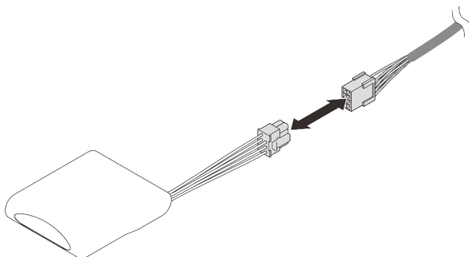
図 76. フラッシュ電源モジュール・ケーブルの接続
