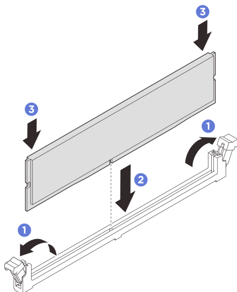
図 174. メモリー・モジュールの取り付け
