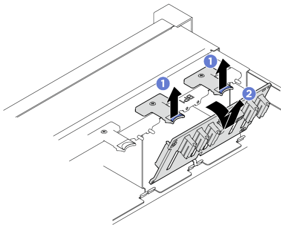
図 24. 2.5 インチ ドライブ・バックプレーンの取り外し
