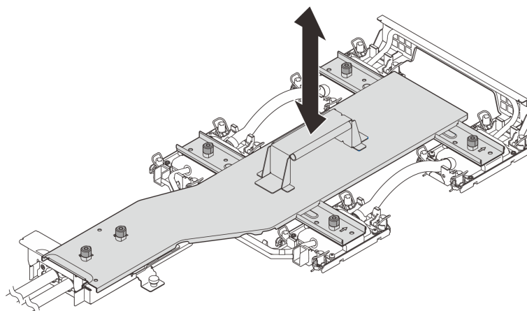
図 111. コールド・プレート・キャリアの取り外し
