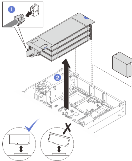
図 182. PCIe LP ライザーの取り外し (電源コネクタあり)
