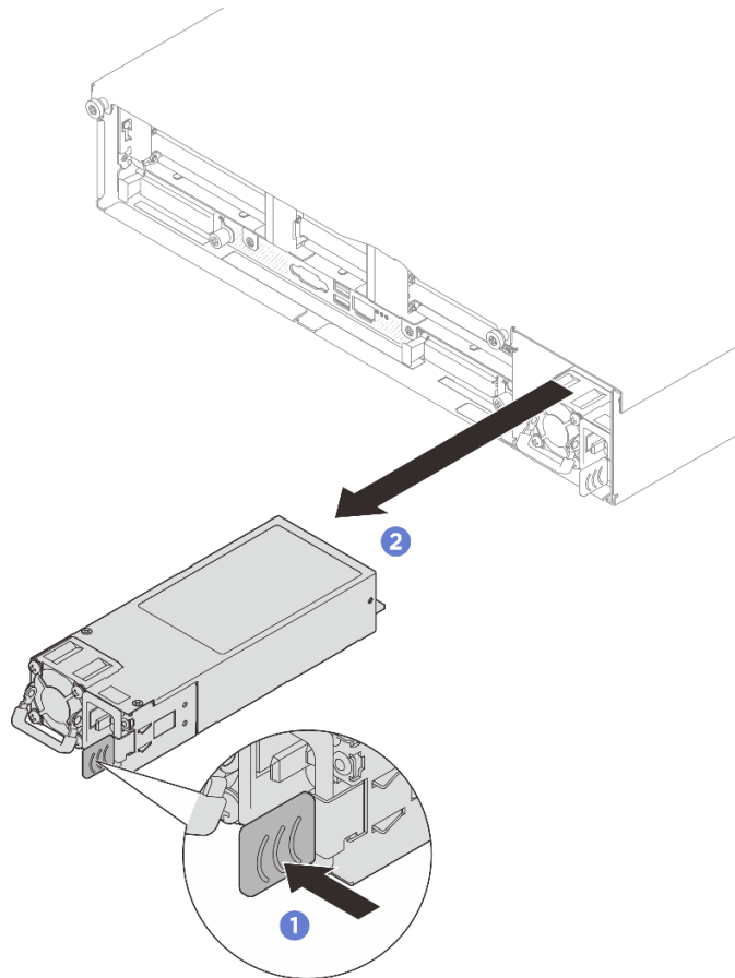
図 207. パワー・サプライ・ユニットの取り外し
