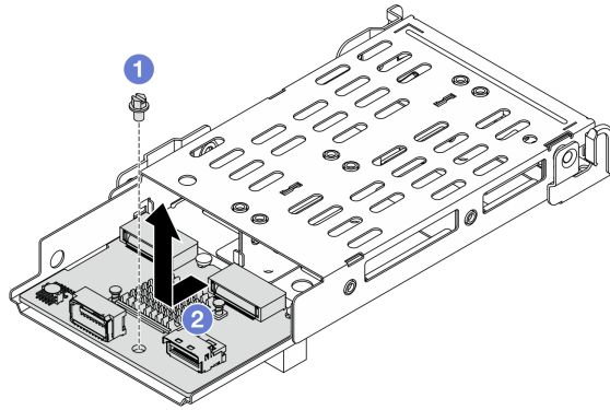
図 227. M.2 ブート・アダプターの取り外し
