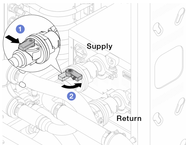
図 129. ボール・バルブを閉じる
