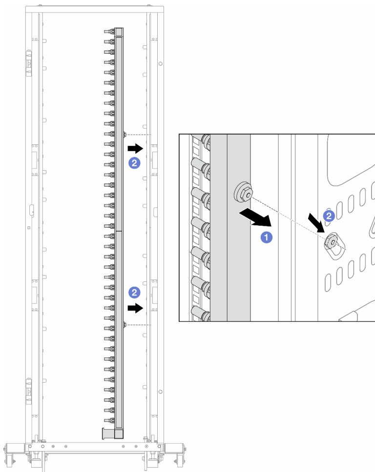
図 160. 多岐管の取り付け
