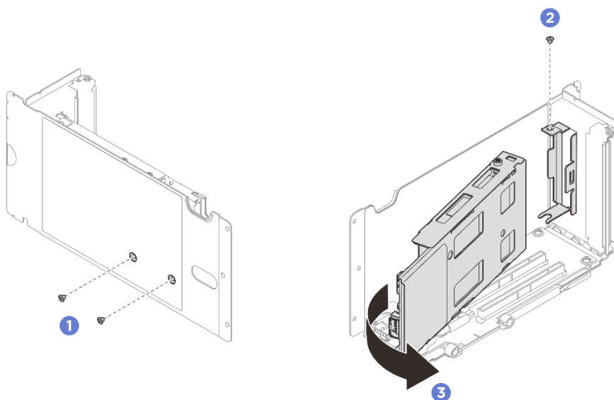
図 226. M.2 ドライブ・ケージの取り外し
