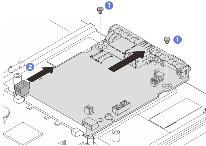
図 248. システム I/O ボードの取り外し
