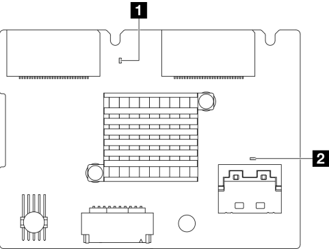
図 270. 背面 M.2 ブート・アダプターの LED
