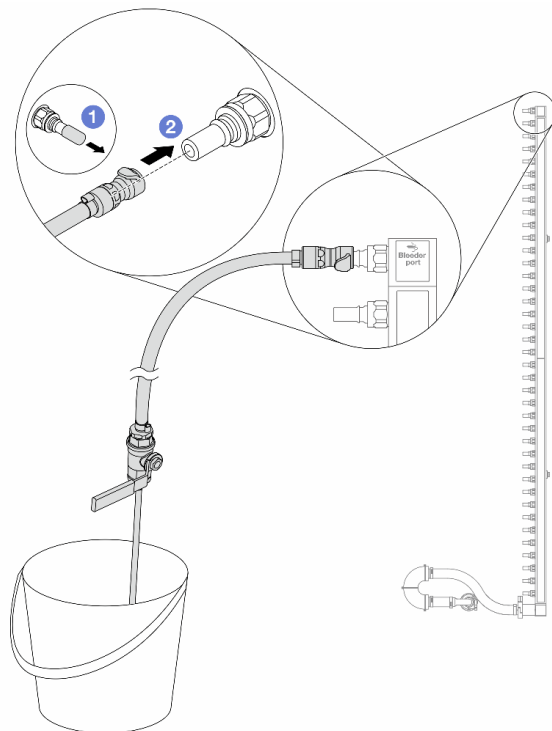
図 135. リターン側へのブリーダー・キットの取り付け
