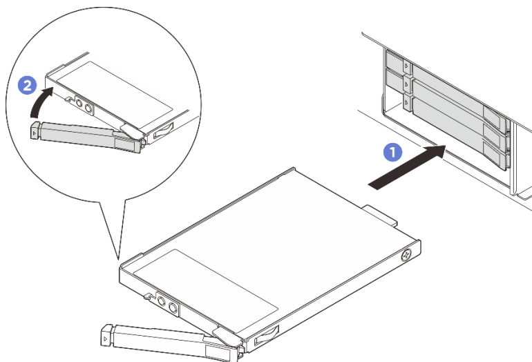
図 60. E3.S ホット・スワップ・ドライブの取り付け
