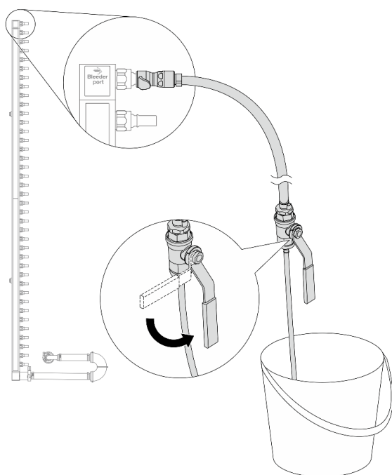
図 134. ブリーダー・バルブを開く
