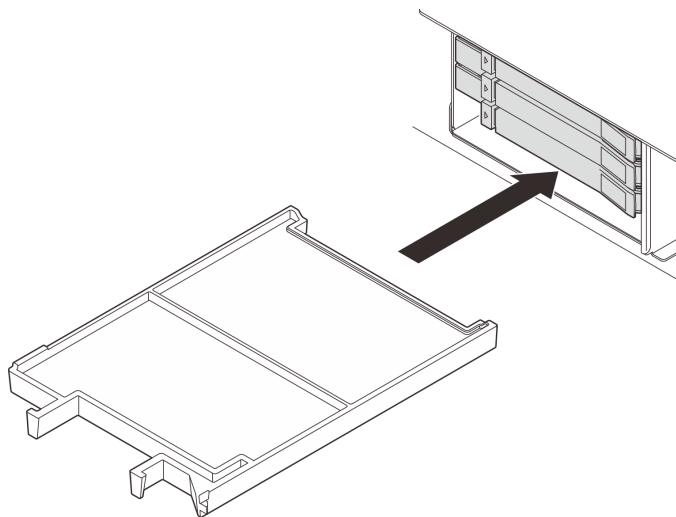
図 61. ベイ・フィラーの取り付け
