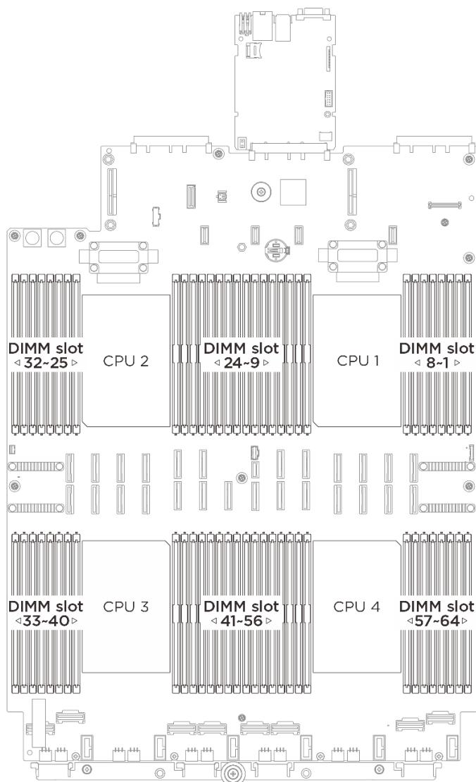
図 173. メモリー・モジュールおよびプロセッサのレイアウト
