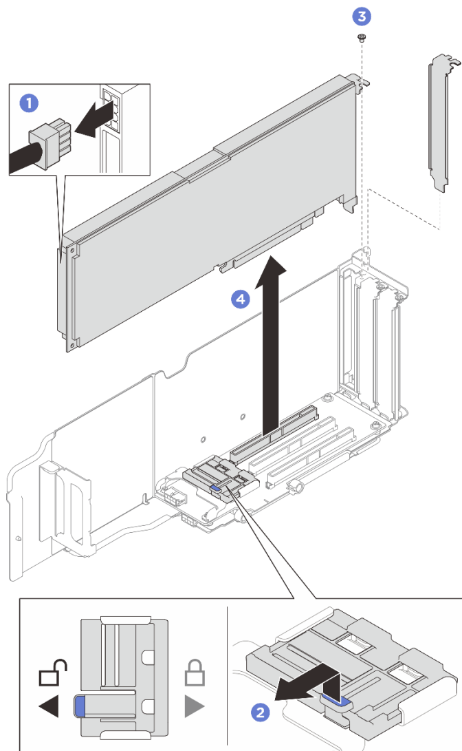
図 77. シングル・ワイド GPU アダプターの取り外し
