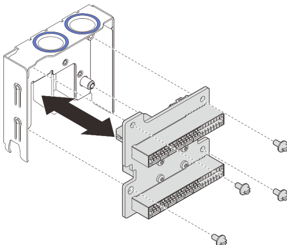
図 205. 分電盤の切り離し
