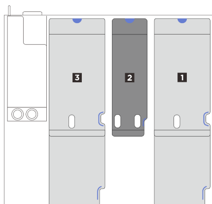
図 188. 3 個の PCIe ライザーおよびライザー・エクステンダーを搭載したサーバー・モデル
