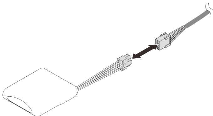
図 72. フラッシュ電源モジュール・ケーブルの切り離し
