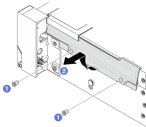
図 220. ケーブル保持具の取り外し
