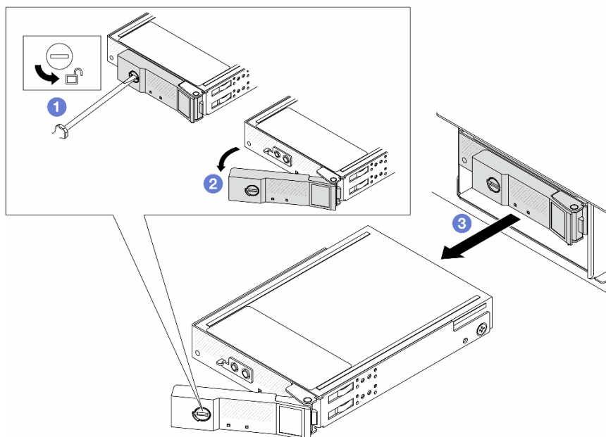
図 44. CMM の取り外し
