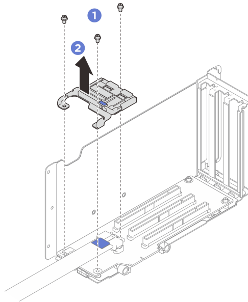
図 200. PCIe 保持具の取り外し
