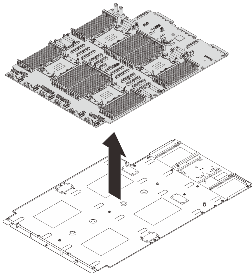
図 280. プロセッサー・ボードの分解
