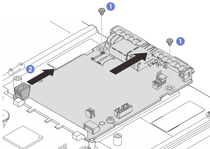
図 277. システム I/O ボードの取り外し
