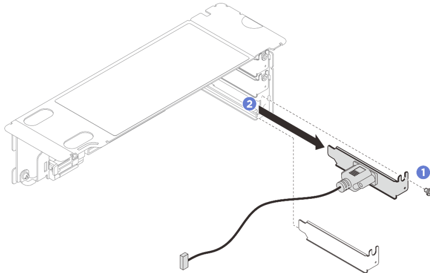
図 237. シリアル・ポート・モジュールの取り外し
