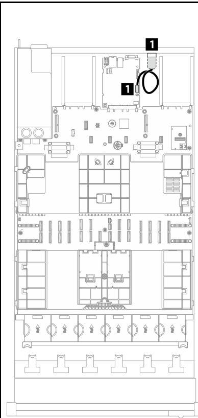
図 241. 4 個の PCIe ライザーを搭載したサーバー・モデルのシリアル・ポート・モジュールのケーブル配線
