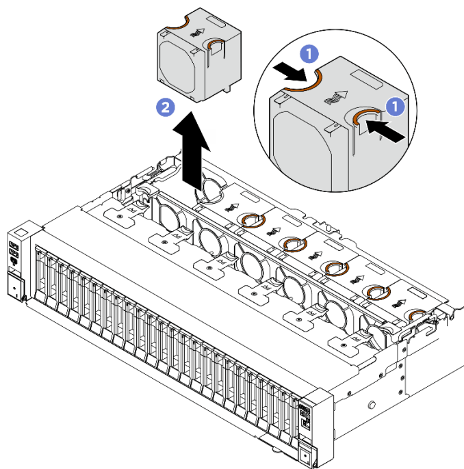
図 68. ファンの取り外し
