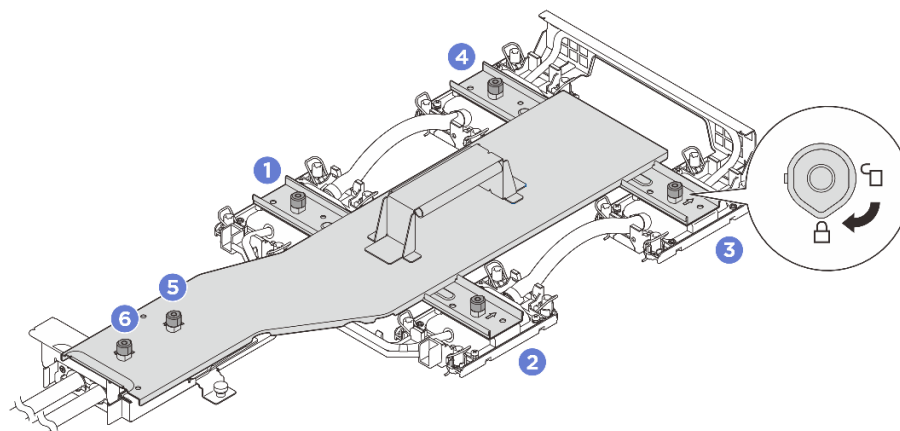
図 100. コールド・プレート・キャリアの固定
