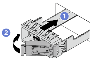
図 83. M.2 ドライブ・トレイの取り付け
