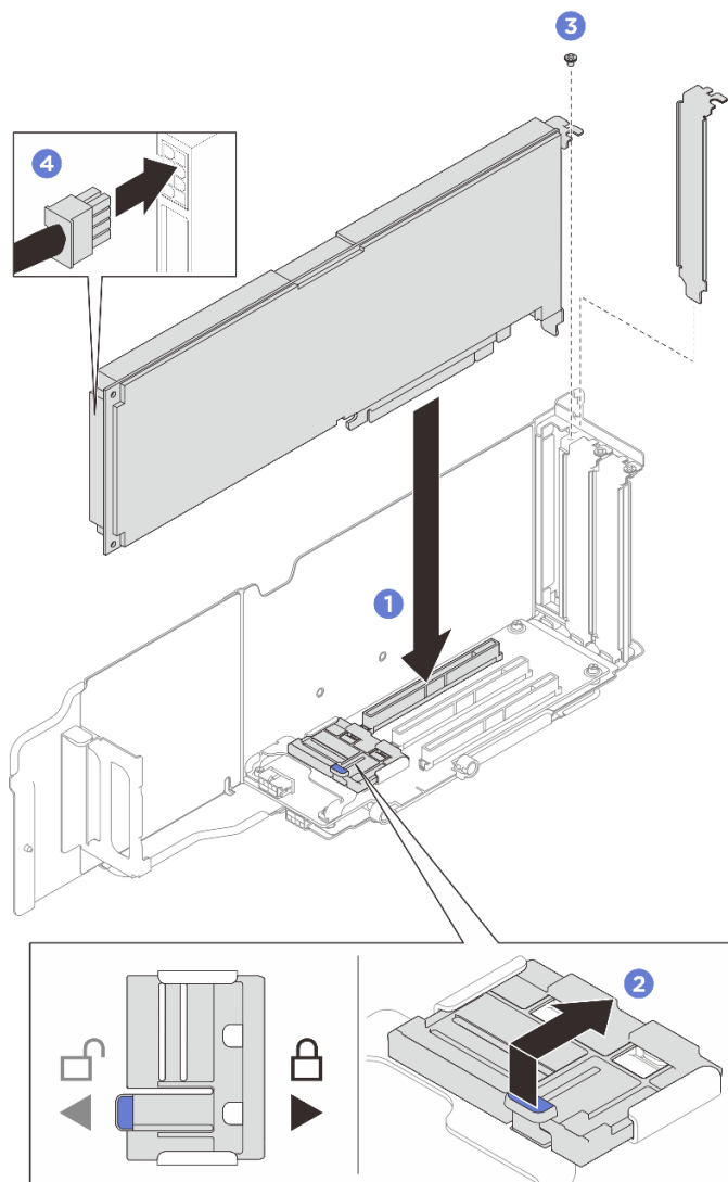
図 79. シングル・ワイド GPU アダプターの取り付け
