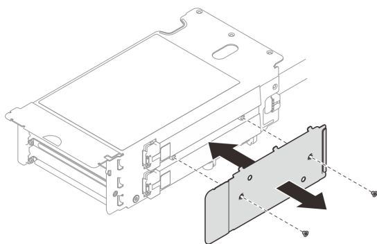
図 199. ケーブル・カバーの取り付け
