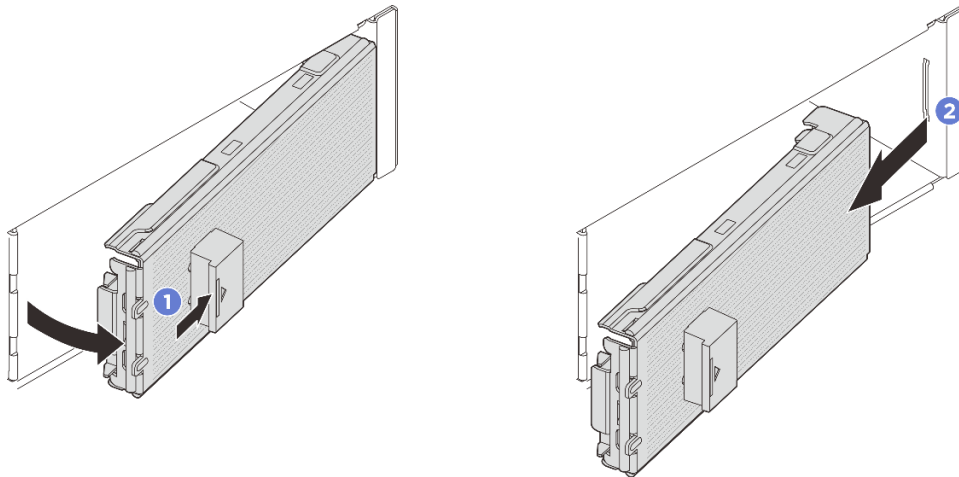
図 46. E3.S ベゼルの取り外し
