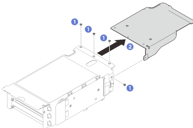
図 202. PCIe ライザー・エクステンダーの取り外し
