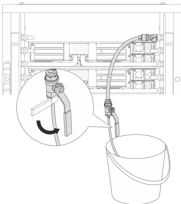
図 168. リターン側のブリーダー・バルブを開く
