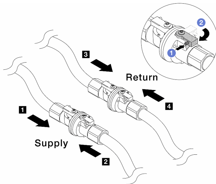
図 170. ボール・バルブを開く
