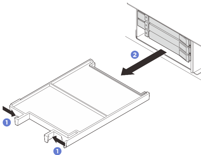
図 59. ベイ・フィラーの取り外し
