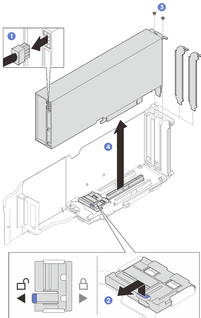
図 78. ダブル・ワイド GPU アダプターの取り外し
