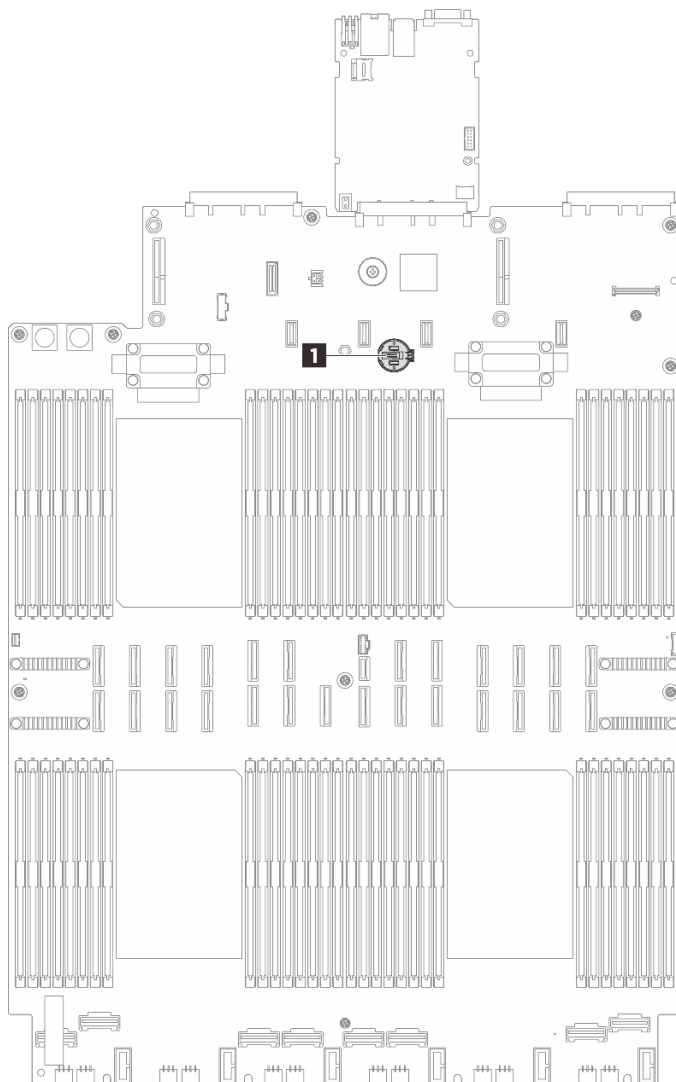
図 39. CMOS バッテリーの位置
