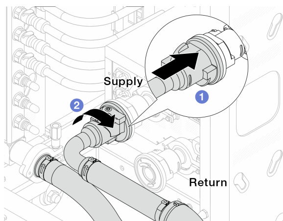
図 142. ボール・バルブの接続
