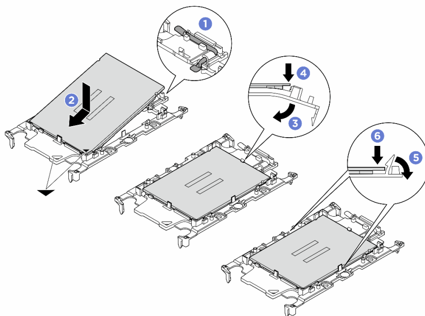
図215. プロセッサ・キャリアの取り付け
