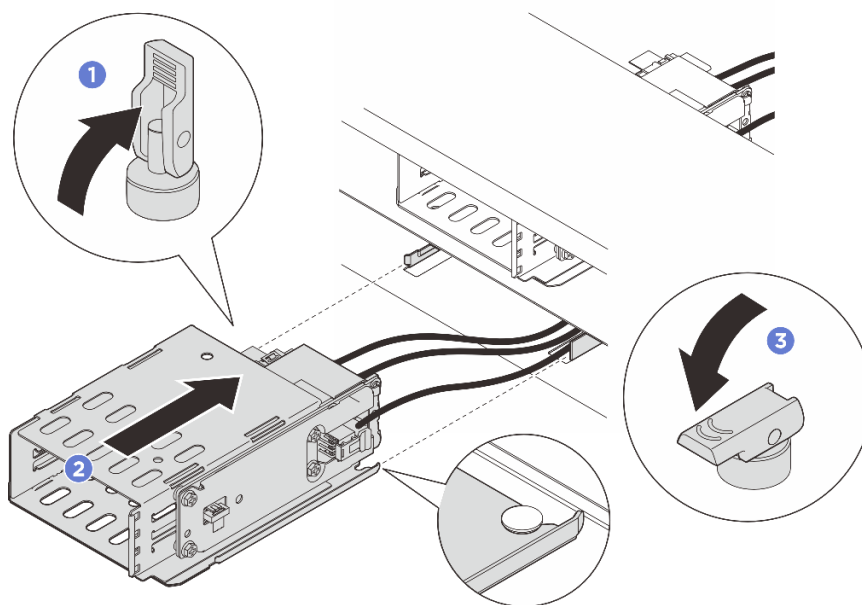
図 67. E3.S 1T ケージの取り付け
