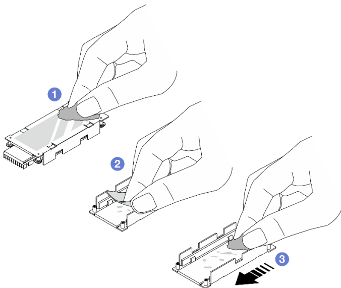
図 87. ヒートシンクと底板のクリーニング
