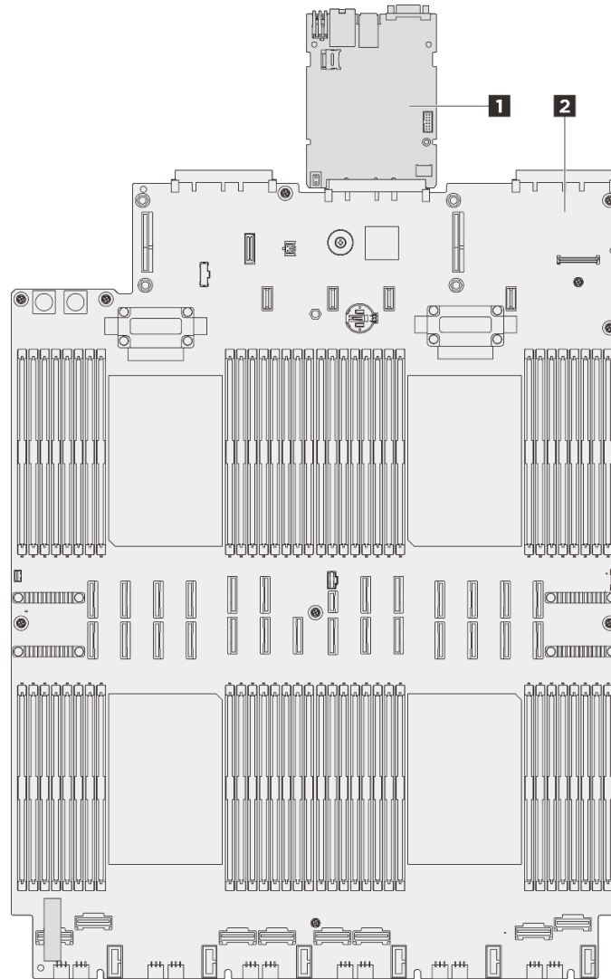
図 242. システム・ボード・アセンブリーのレイアウト
