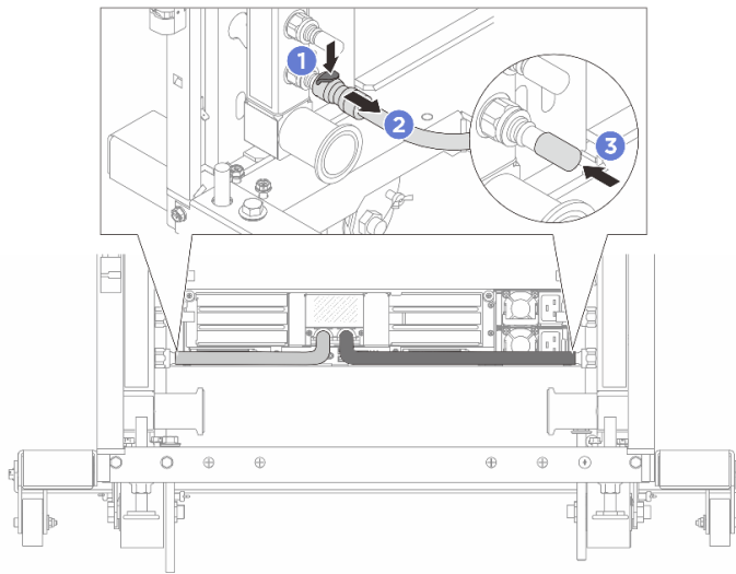
図 153. クイック・コネクト・プラグの取り外し
