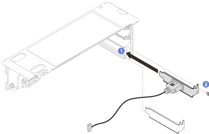
図238. シリアル・ポート・モジュールの取り付け
