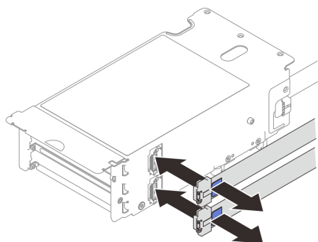
図 198. ケーブル配線
