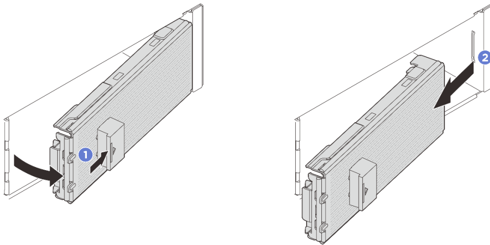
図 58. E3.S ベゼルの取り外し
