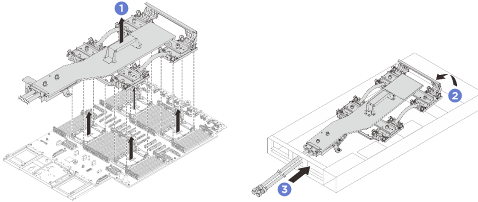
그림 84. 냉각판 어셈블리 제거
