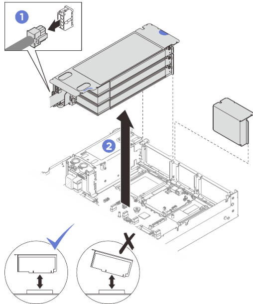
그림 163. PCIe LP 라이저 제거(전원 커넥터 포함)
