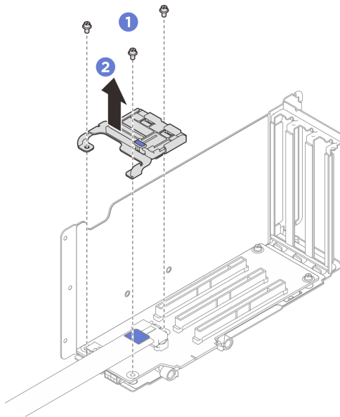
그림 181. PCIe 고정장치 제거
