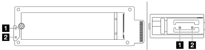
그림 251. 뒷면 M.2 인터포저 LED
