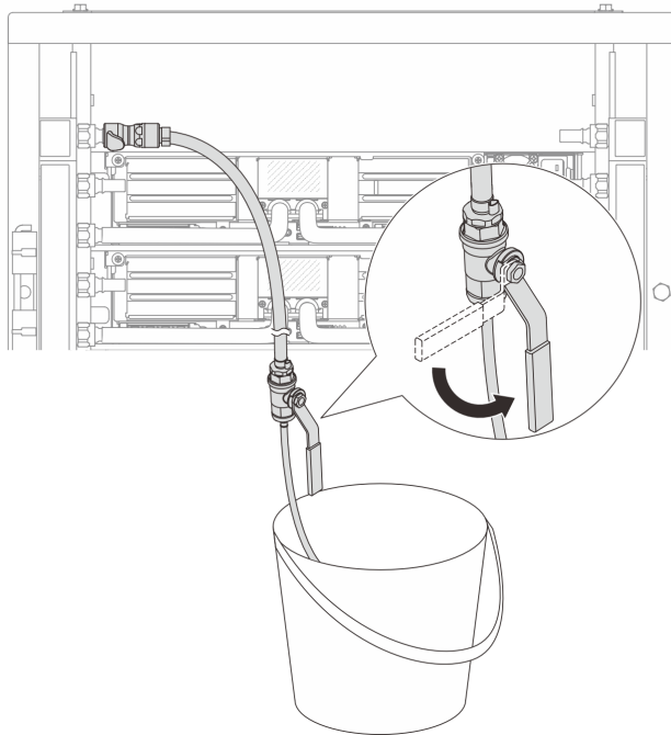
그림 129. 공급 측 블리드 밸브 열기
