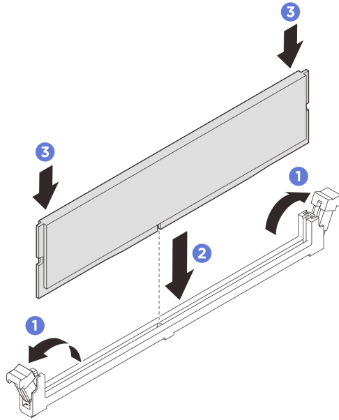
그림 155. 메모리 모듈 설치
