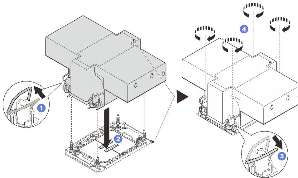
그림 200. 2U 성능 PHM 설치
