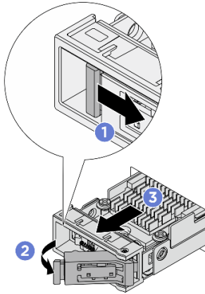
그림 63. 핫 스왑 M.2 드라이브 어셈블리 제거
