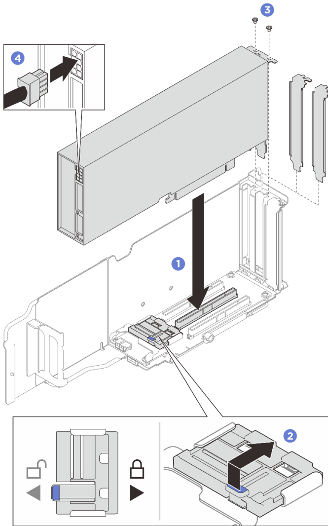
그림 61. 더블 와이드 GPU 어댑터 설치
