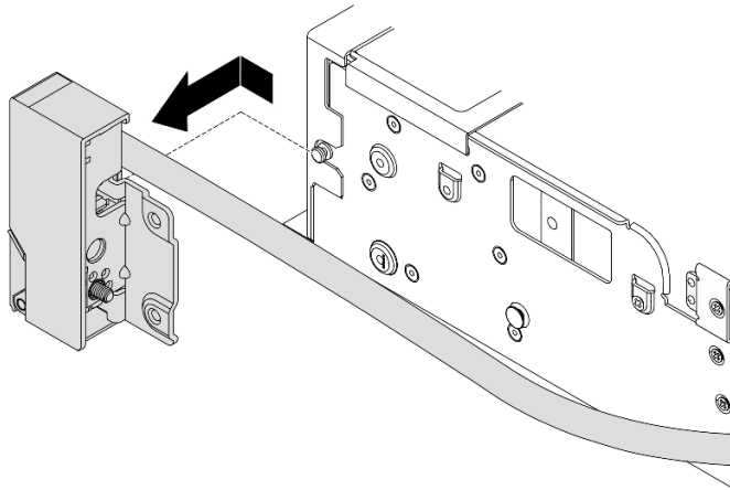
그림 203. 랙 래치 제거
