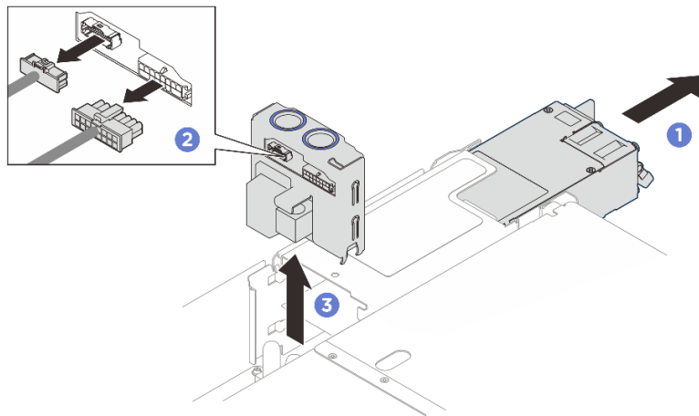
그림 185. 전원 분배 보드 제거
