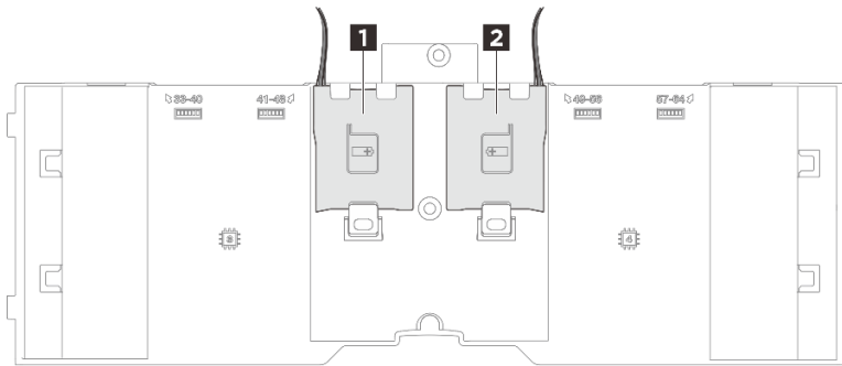
그림 55. 플래시 전원 모듈 슬롯 위치
