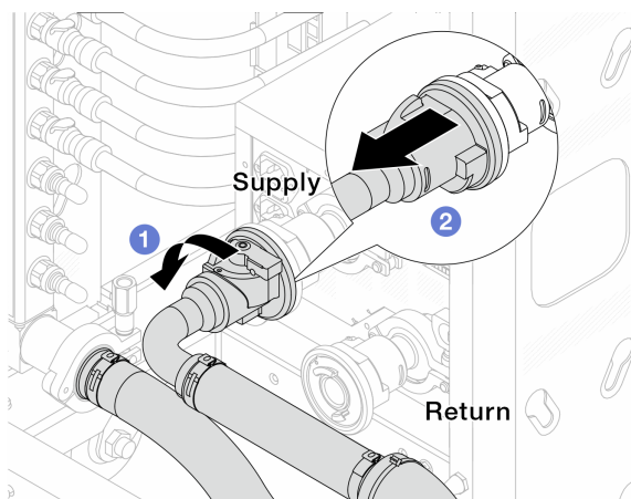
그림 112. 연결 세트 제거
