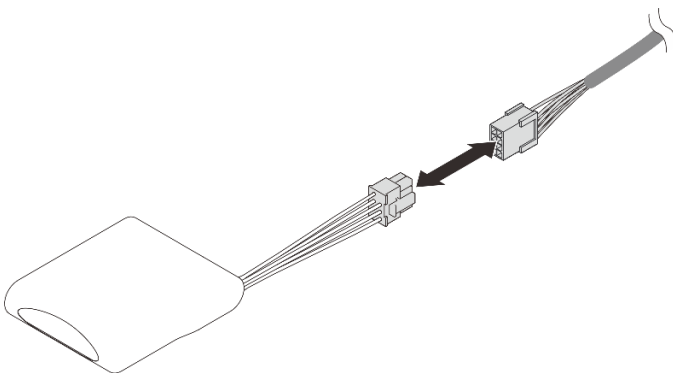
그림 19. 플래시 전원 모듈 케이블 연결
