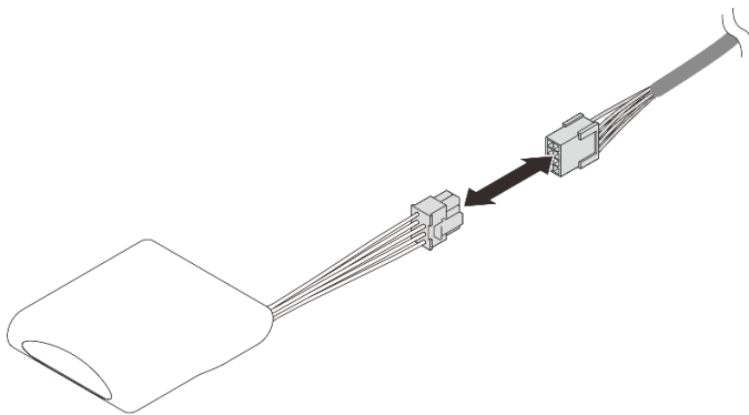
그림 8. 플래시 전원 모듈 케이블 분리
