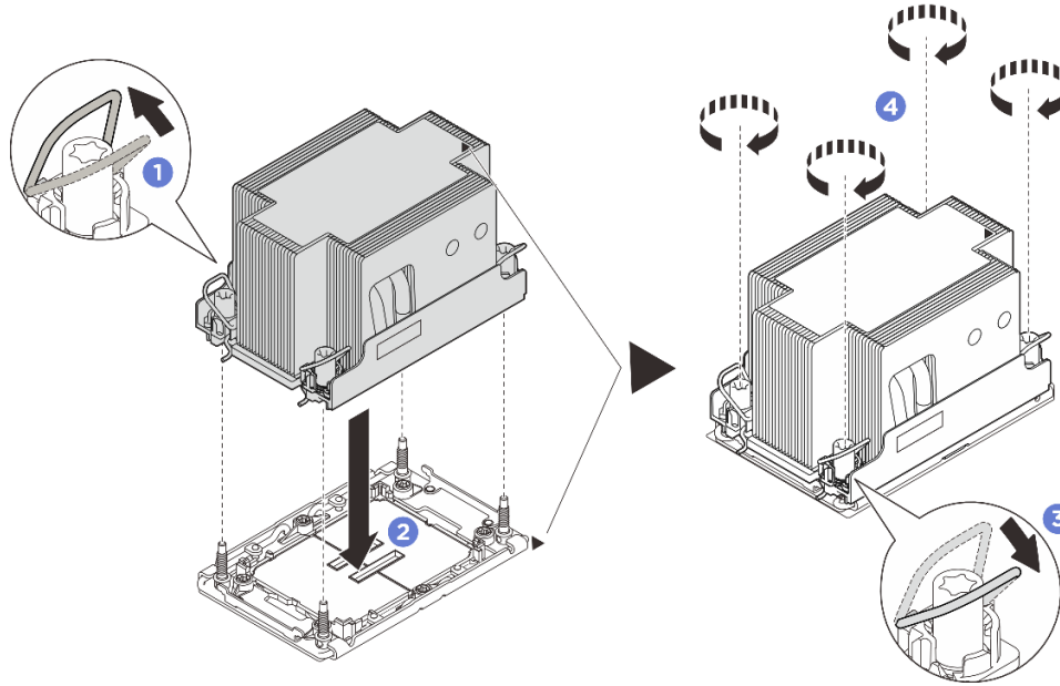
그림 199. 2U 표준 PHM 설치
