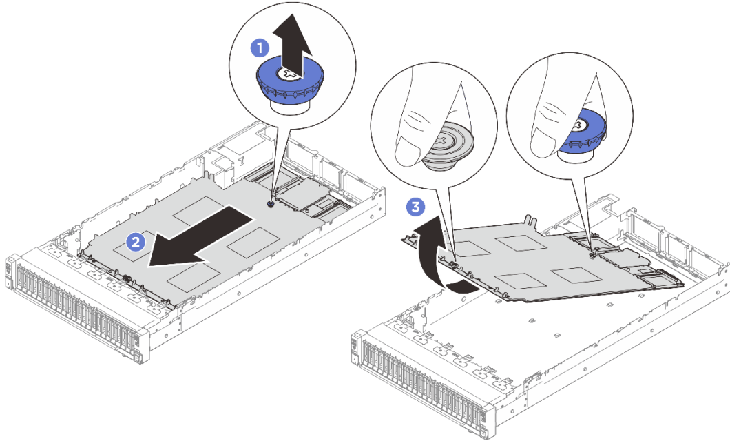
그림 228. 시스템 보드 어셈블리 제거
