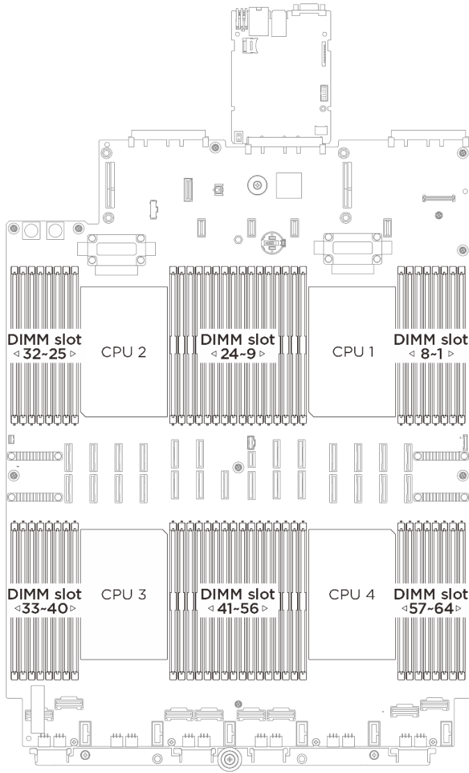
그림 152. 메모리 모듈 및 프로세서 레이아웃
