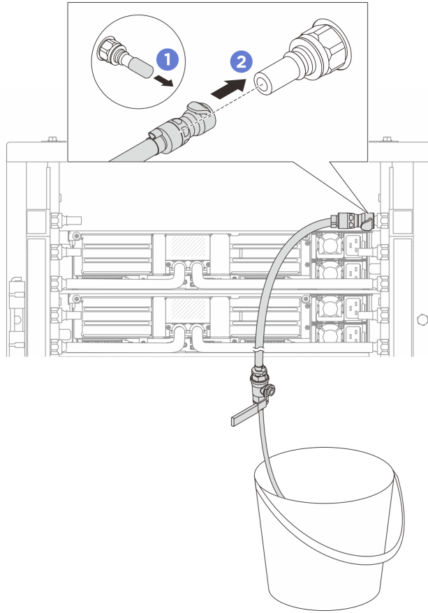
그림 130. 리턴 측에 블리드 키트 설치
