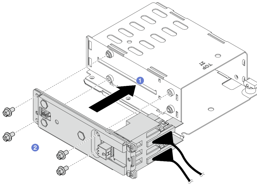
그림 35. 백플레인 설치
