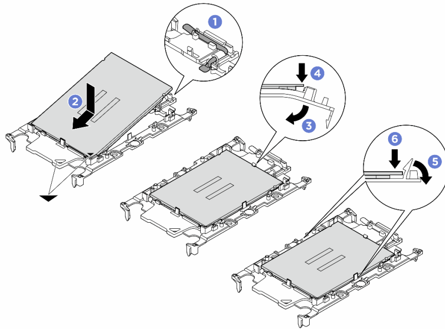
그림 196. 프로세서 캐리어 설치
