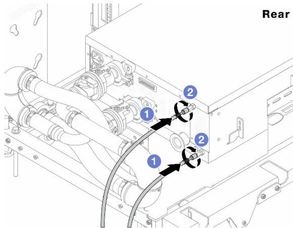
그림 125. CDU 뒷면
