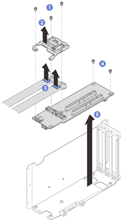
그림 176. PCIe 라이저 카드 제거
