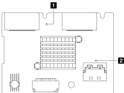
그림 252. 뒷면 M.2 부트 어댑터 LED
