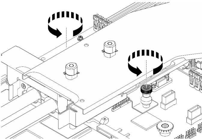
그림 83. 냉각팬 어셈블리 제거
