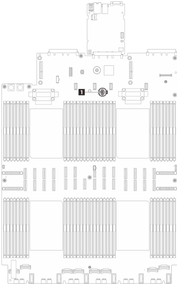
그림 22. CMOS 배터리 소켓 위치
