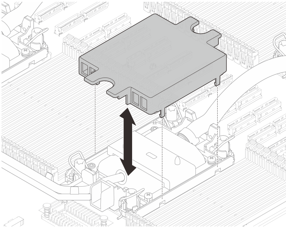
그림 258. 냉각판 덮개 제거
