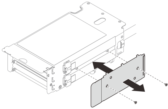
그림 180. 케이블 덮개 설치
