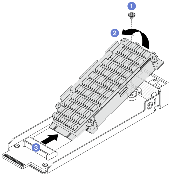
그림 65. 방열판이 있는 M.2 드라이브 제거
