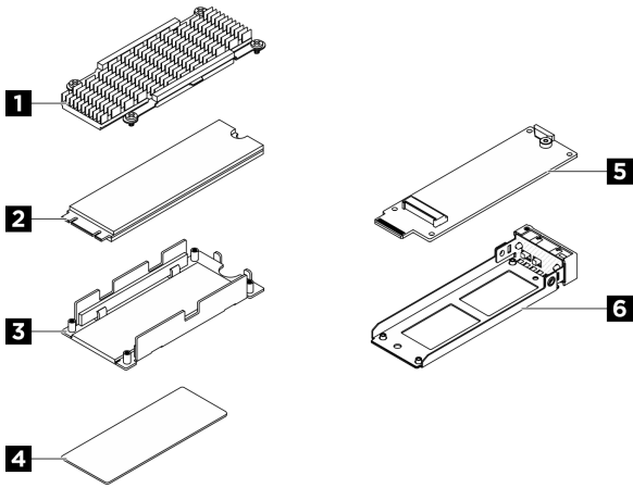
그림 62. 핫 스왑 M.2 드라이브 어셈블리의 부품
