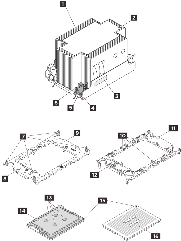
그림 195. PHM 구성 요소
