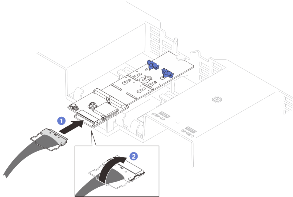
그림 100. M.2 부트 어댑터 케이블 연결
