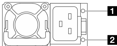
그림 248. CRPS Premium(CFFv5) 전원 공급 장치의 LED
