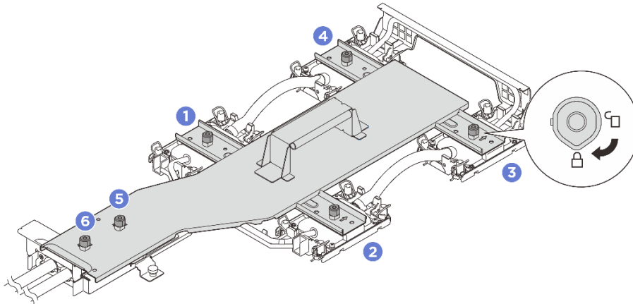
그림 81. 냉각판 캐리어 고정
