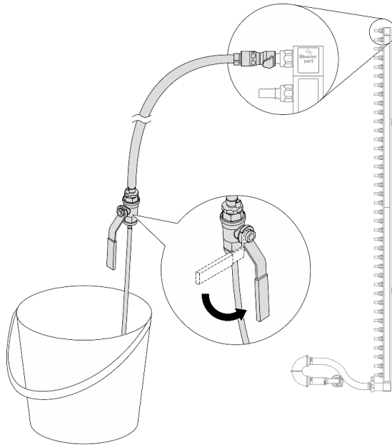
그림 117. 블리드 밸브 열기
