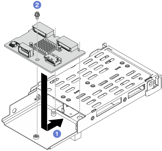
그림 209. M.2 부트 어댑터 설치
