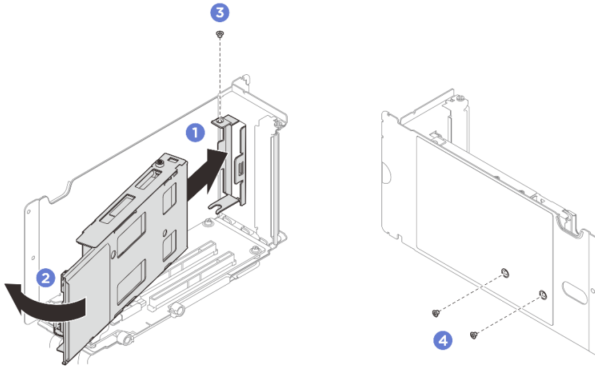
그림 210. M.2 드라이브 케이스 설치
