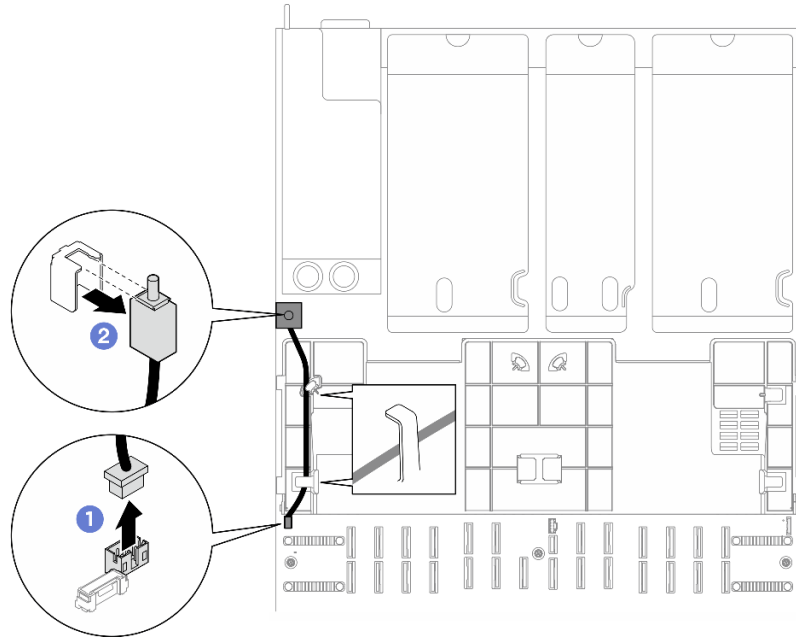
그림 75. 침입 스위치 제거
