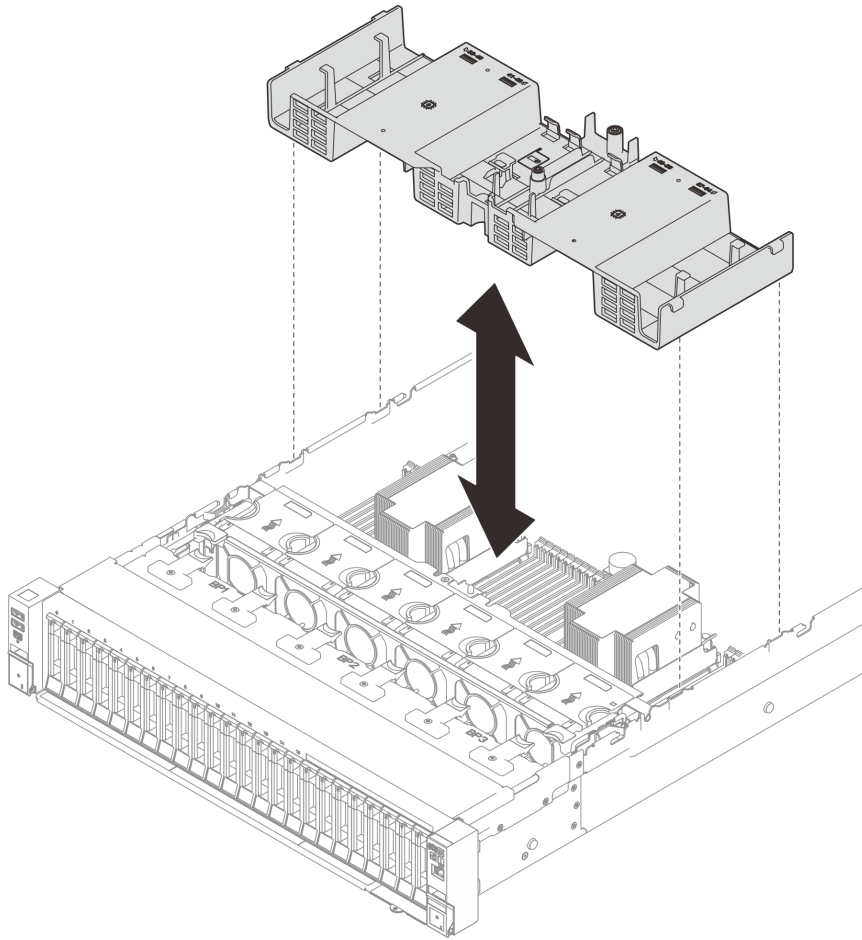
그림 10. 전면 공기 조절 장치 제거
