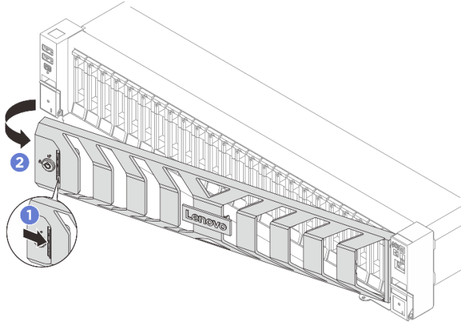
그림 214. 보안 베젤 제거
