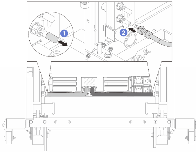
그림 142. 퀵 커넥트 플러그 설치
