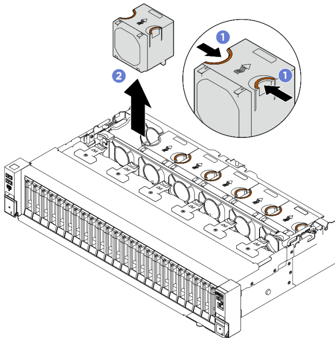
그림 49. 팬 제거
