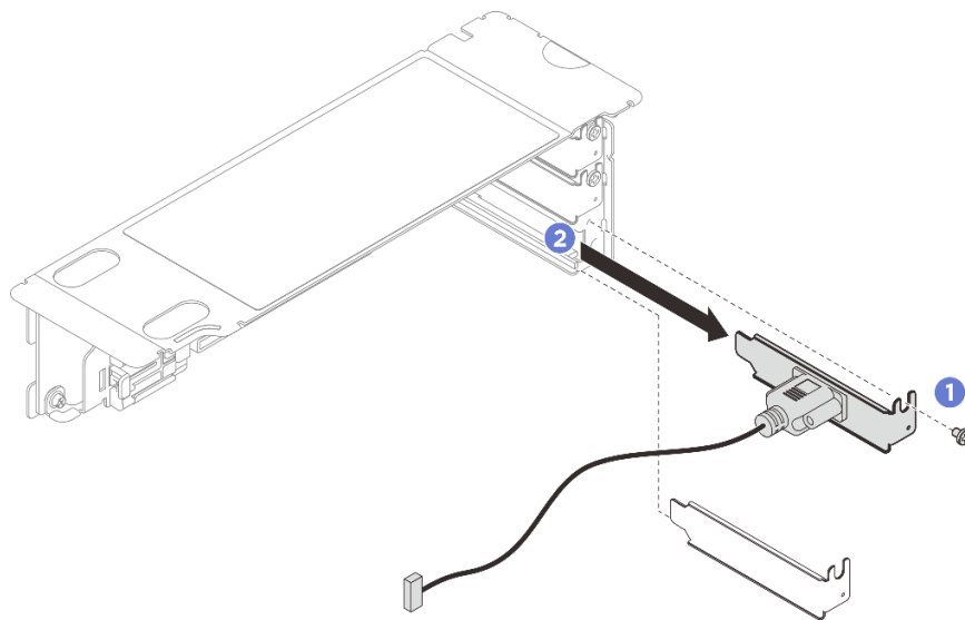
그림 218. 직렬 포트 모듈 제거
