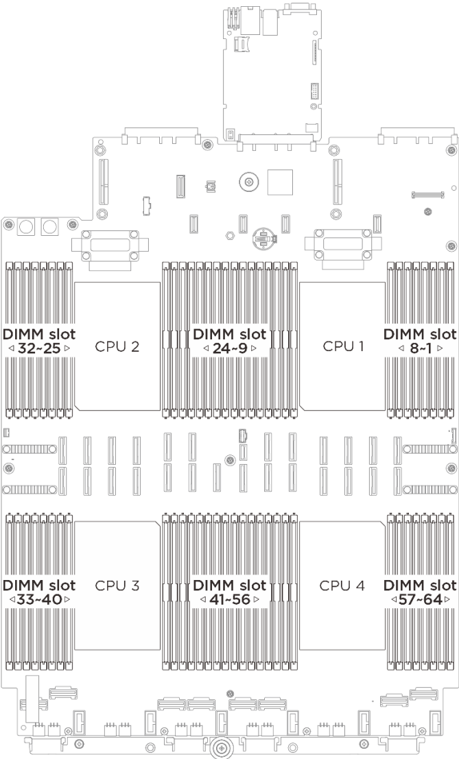
그림 1. 메모리 모듈 및 프로세서 레이아웃
