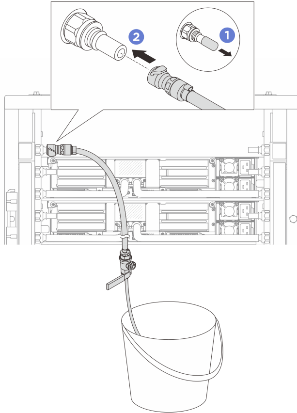
그림 144. 공급 측에 블리드 키트 설치
