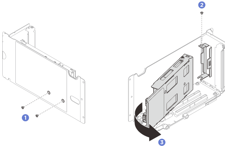
그림 207. M.2 드라이브 케이지 제거
