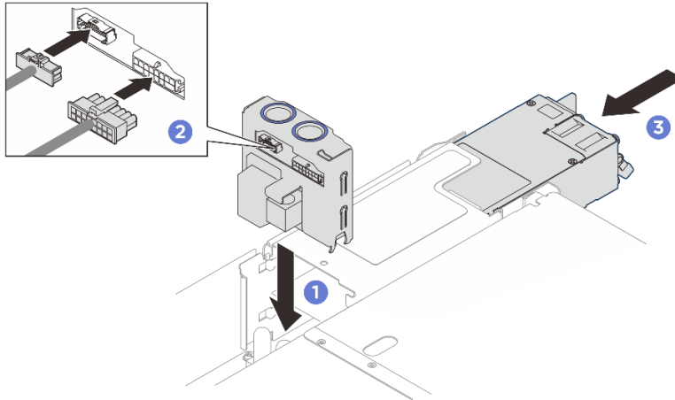
그림 187. 전원 분배 보드 설치
