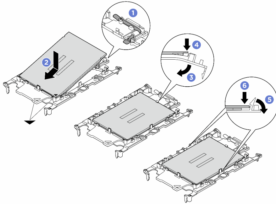
그림 85. 프로세서 캐리어 설치
