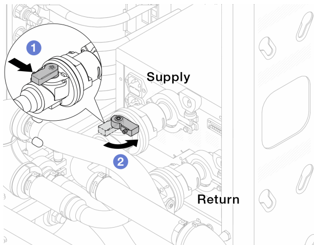
그림 110. 볼 밸브 닫기
