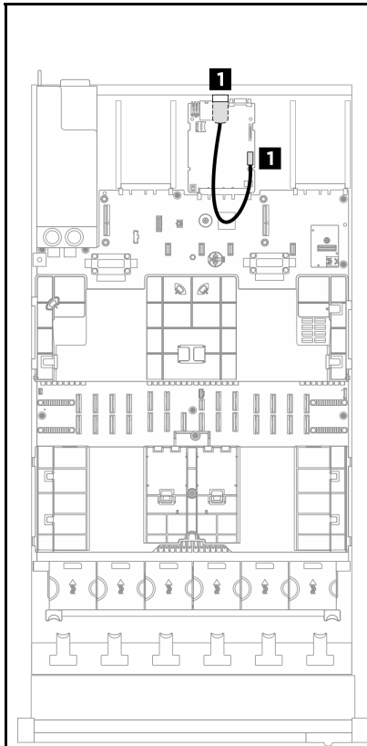
그림 221. PCIe 라이저 3개가 지원되는 서버 모델의 직렬 포트 모듈 케이블 배선
