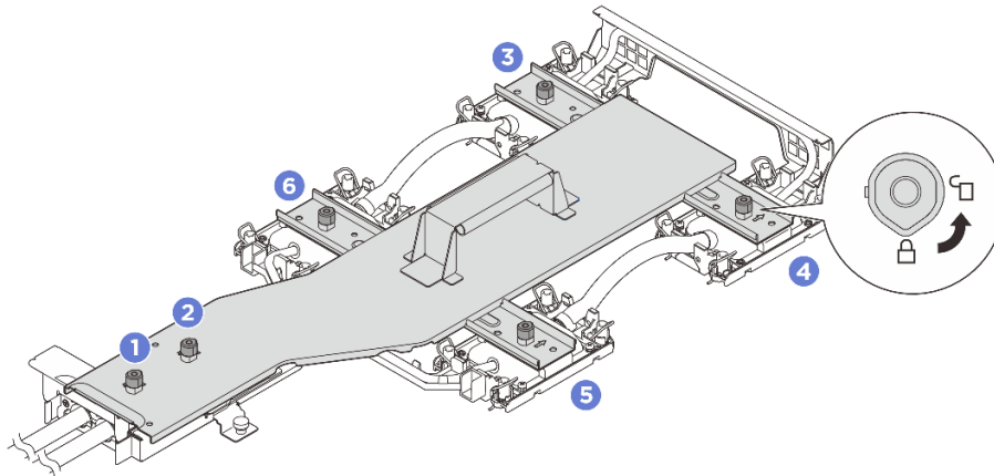
그림 91. 냉각판 캐리어 풀기
