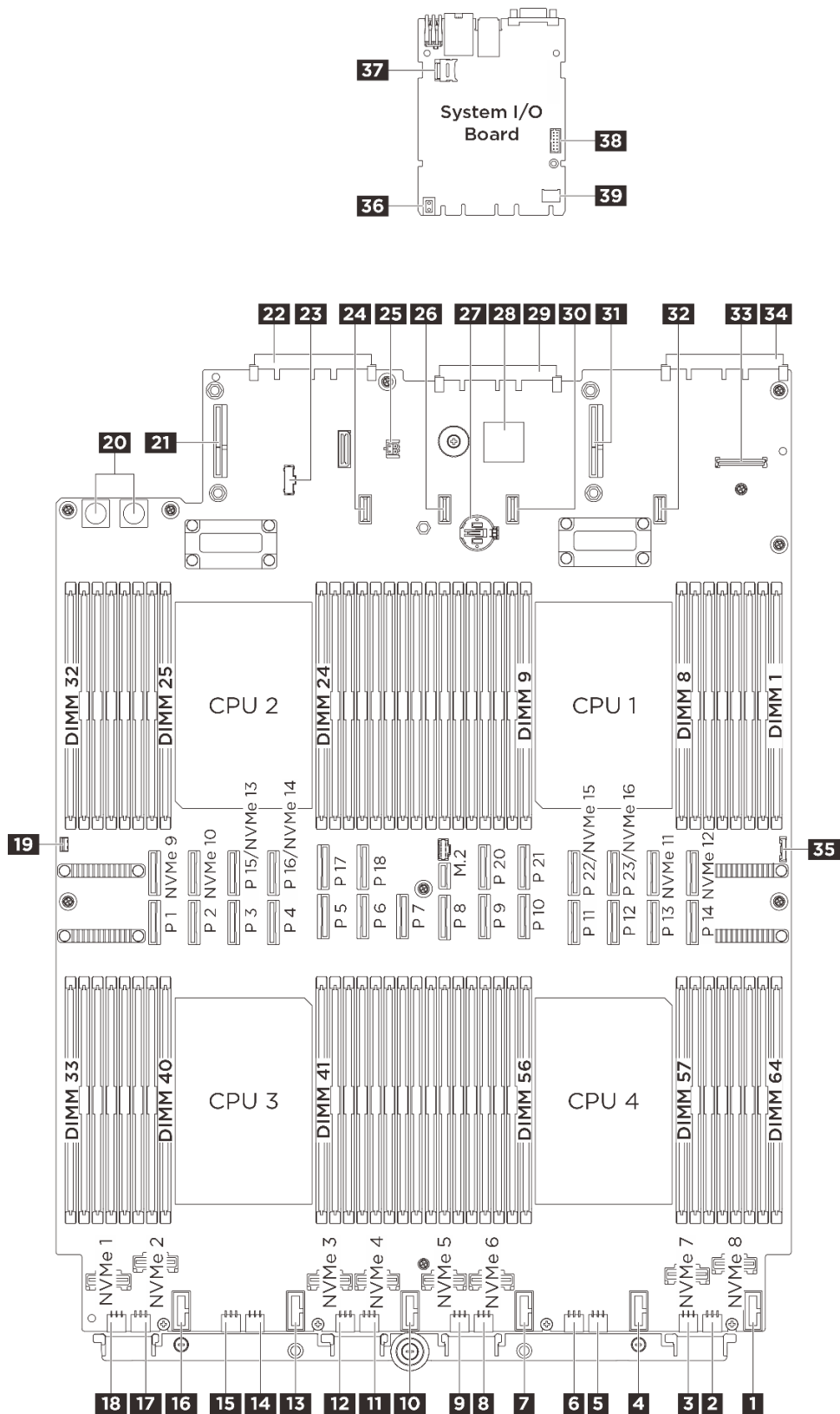
그림 242. 시스템 보드 어셈블리 커넥터
