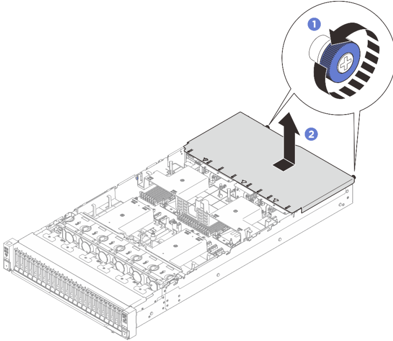
그림 234. 뒤쪽 윗면 덮개 제거
