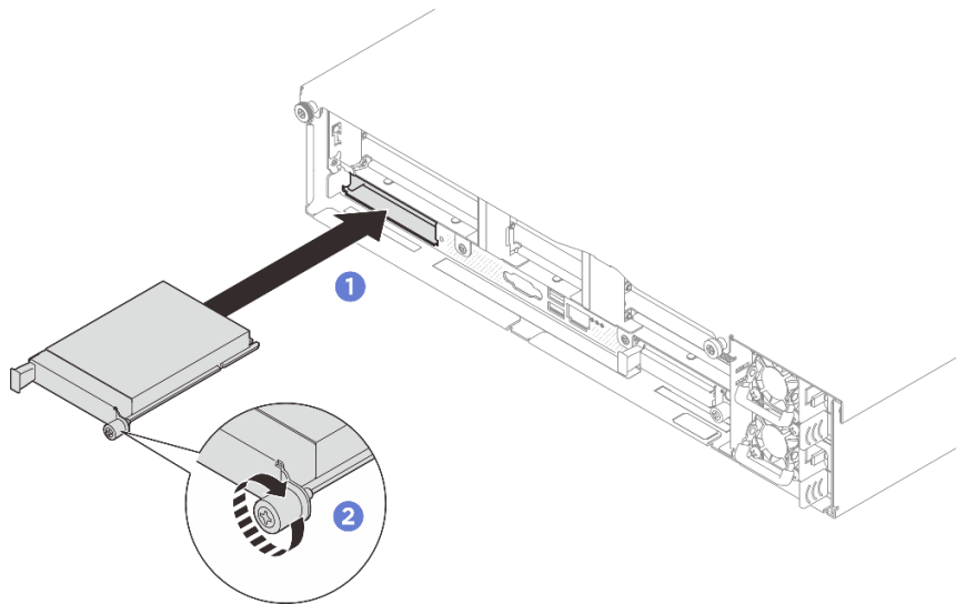
그림 159. OCP 모듈 설치
