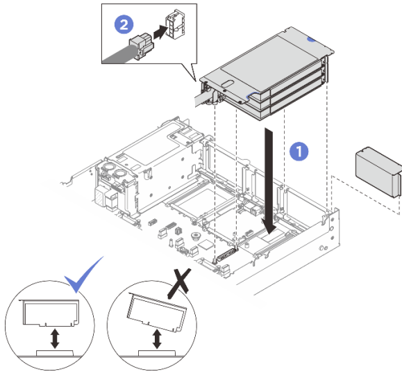
그림 172. PCIe FHHL 라이저 설치
