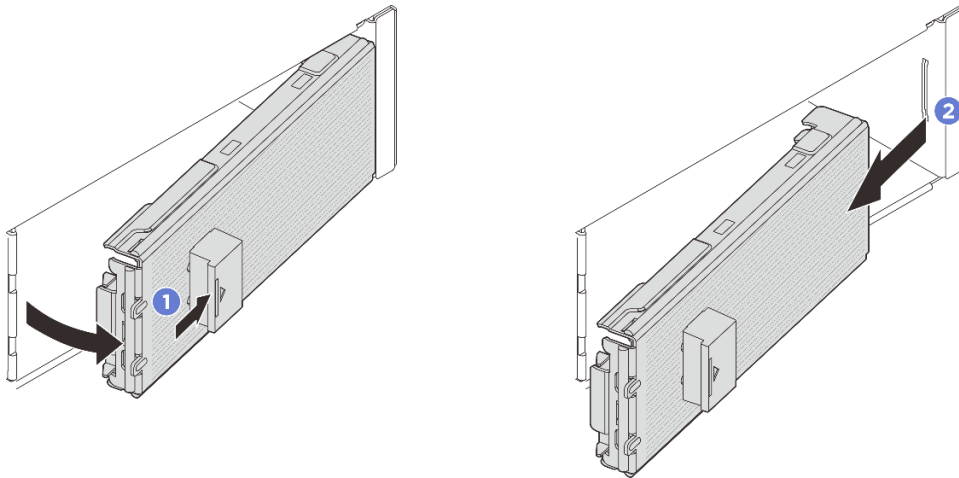
그림 27. E3.S 베젤 제거
