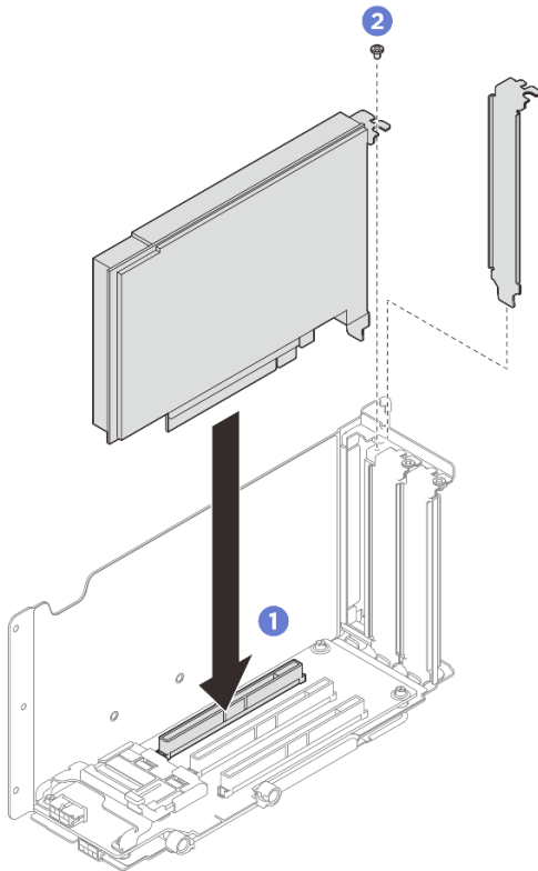
그림 167. PCIe 어댑터 설치
