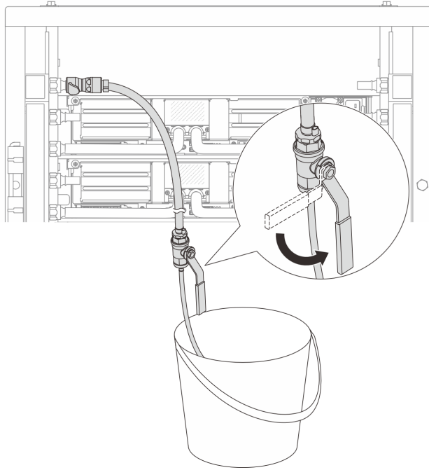
그림 146. 공급 측 블리드 밸브 열기
