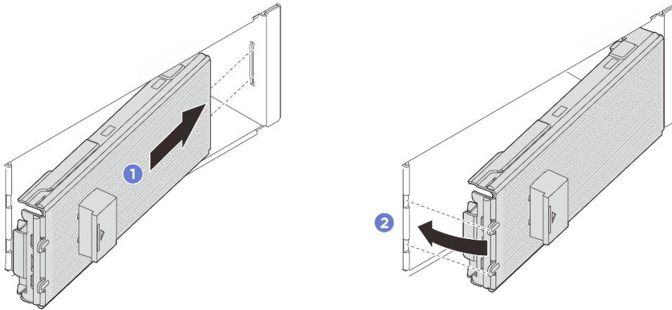
그림 32. E3.S 베젤 설치
