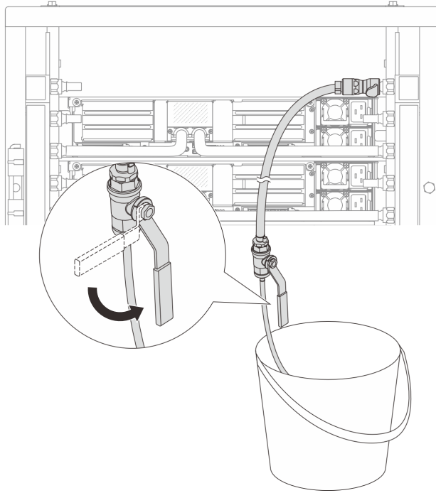
그림 131. 리턴 측 블리드 밸브 열기
