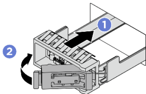
그림 64. M.2 드라이브 트레이 설치
