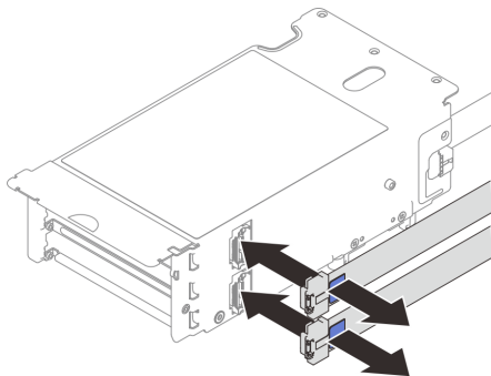
그림 175. 케이블 분리
