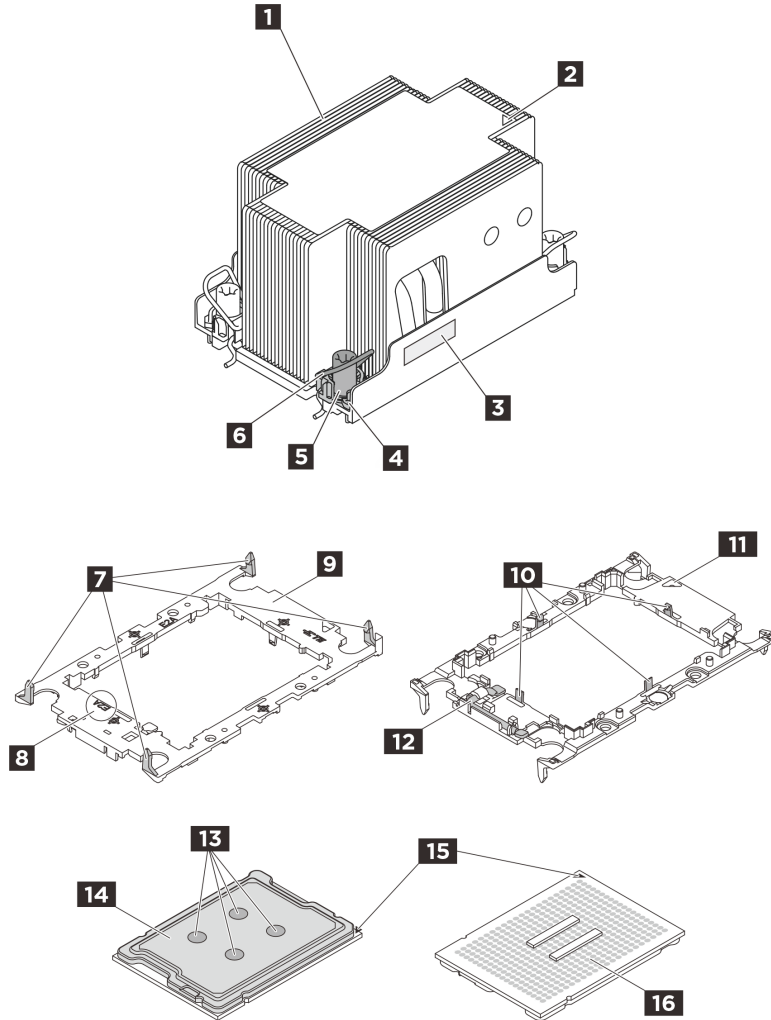
그림 190. PHM 구성 요소
