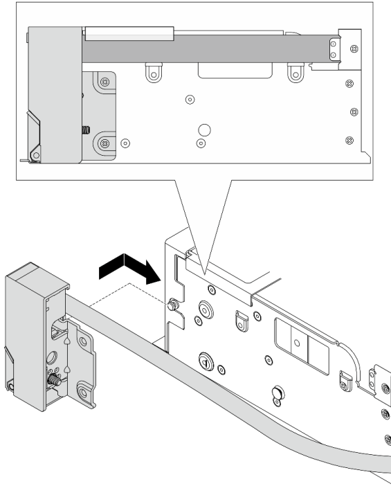
그림 204. 랙 래치 설치
