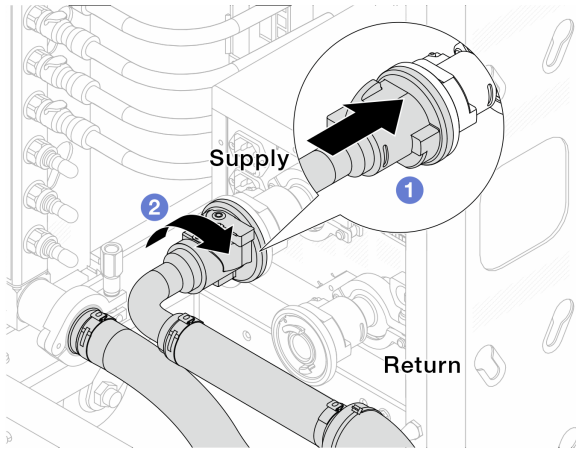
그림 123. 볼 밸브 연결
