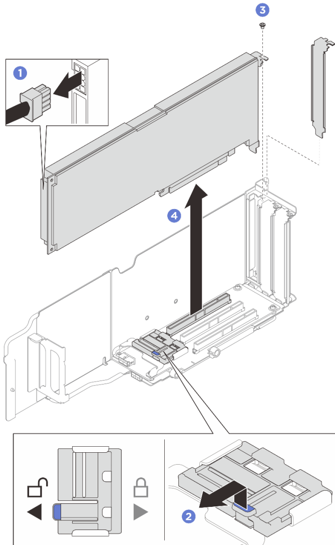
그림 58. 싱글 와이드 GPU 어댑터 제거
