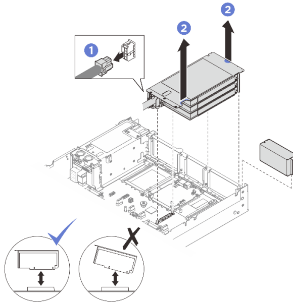
그림 164. PCIe FHFL 라이저 제거
