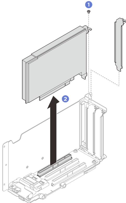
그림 166. PCIe 어댑터 제거
