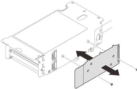
그림 177. 케이블 덮개 제거
