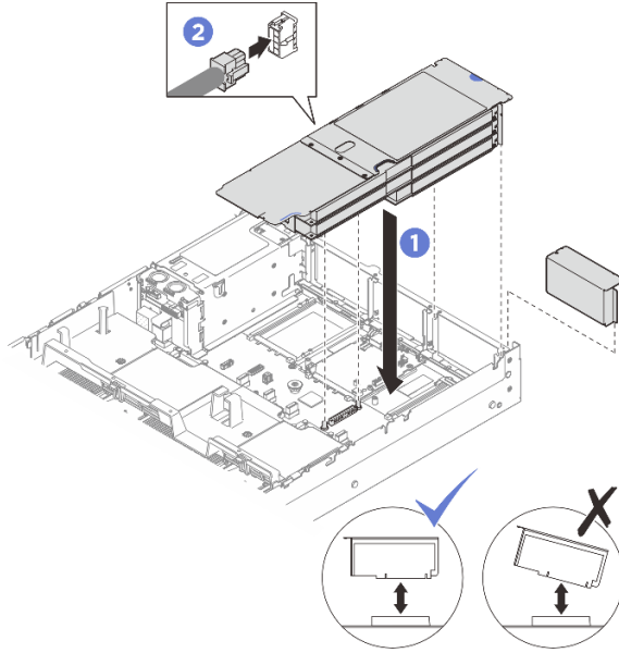
그림 173. PCIe FHFL 라이저 설치
