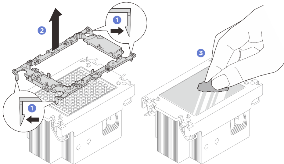
그림 194. 방열판에서 프로세서 캐리어 분리 중
