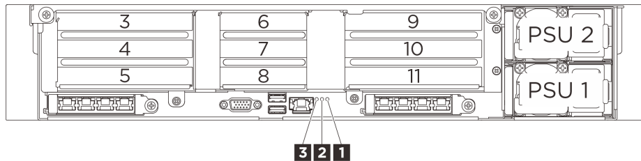
그림 253. 뒷면 시스템 LED
