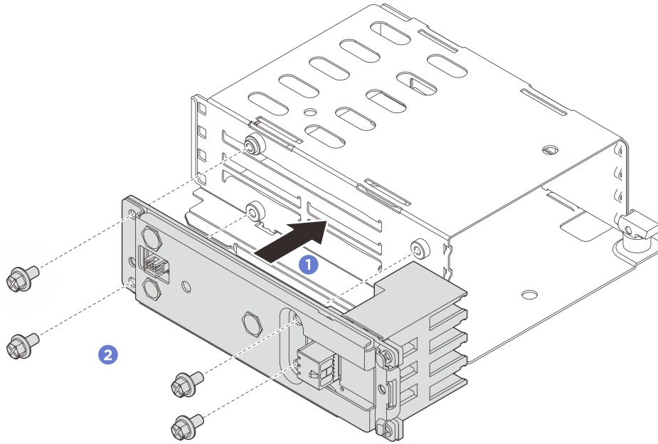
그림 47. 백플레인 어셈블리 설치
