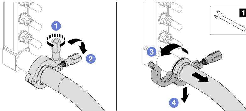
그림 118. 연결 세트에서 매니폴드 분리
