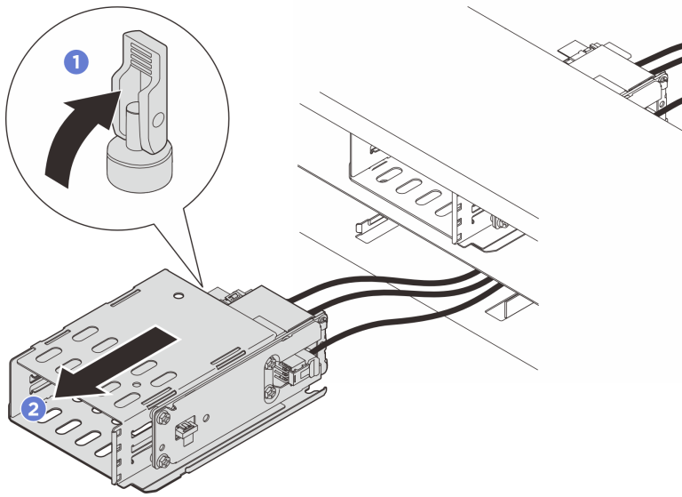
그림 45. E3.S 1T 케이지 제거
