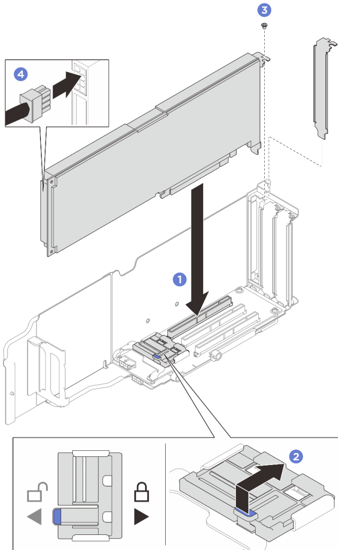
그림 60. 싱글 와이드 GPU 어댑터 설치
