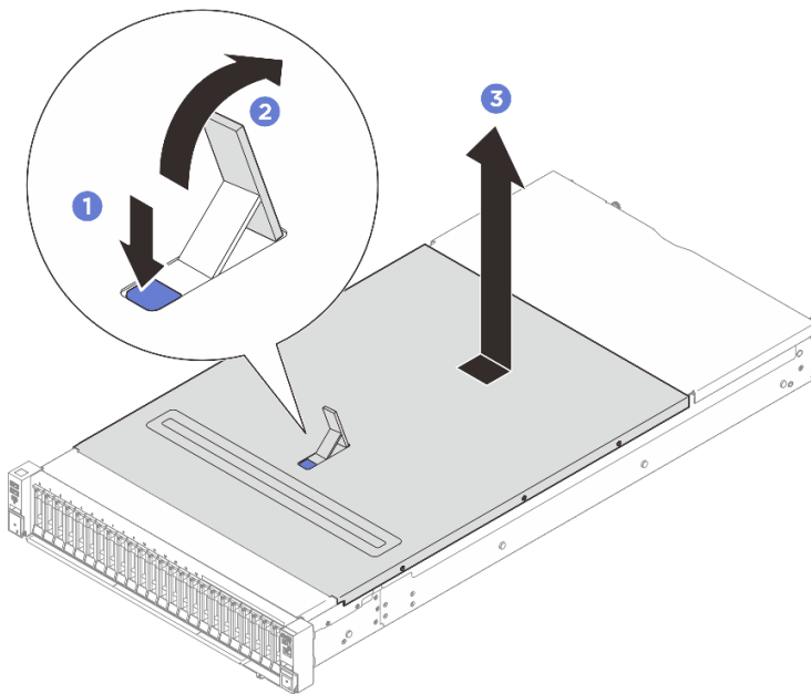
그림 233. 앞쪽 윗면 덮개 제거
