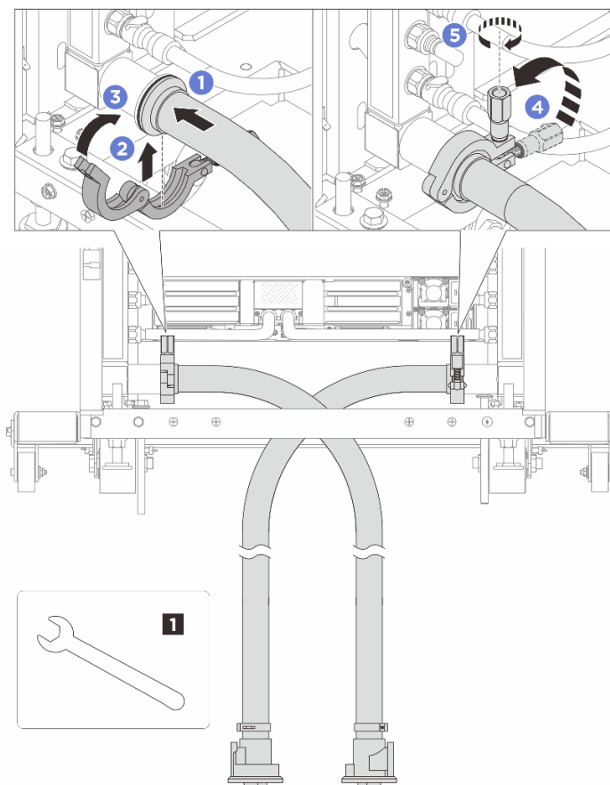
그림 143. 호스 키트 설치
