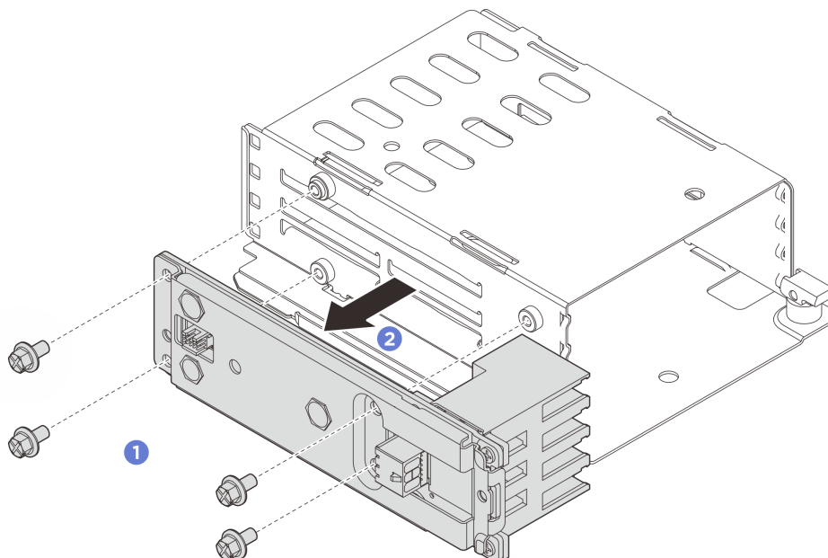
그림 46. 백플레인 어셈블리 제거
