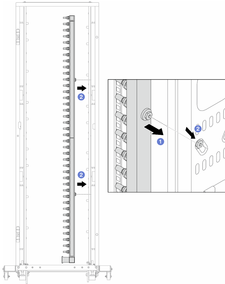
그림 141. 매니폴드 설치
