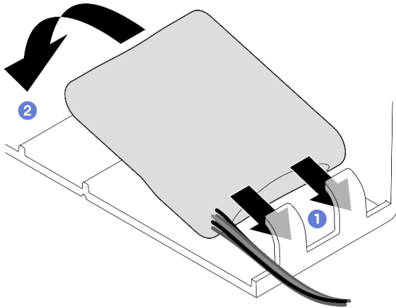
그림 56. 플래시 전원 모듈 설치
