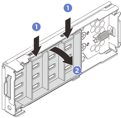
그림 31. 내부 플레이트 제거
