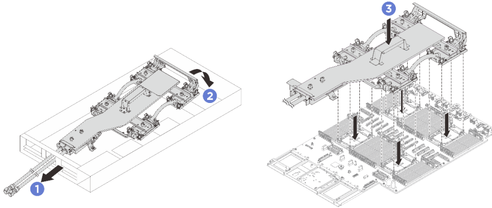
그림 88. 냉각판 어셈블리 설치
