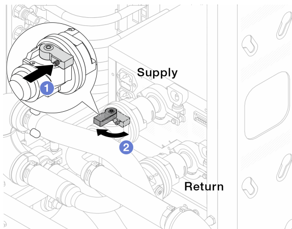
그림 128. 볼 밸브 열기
