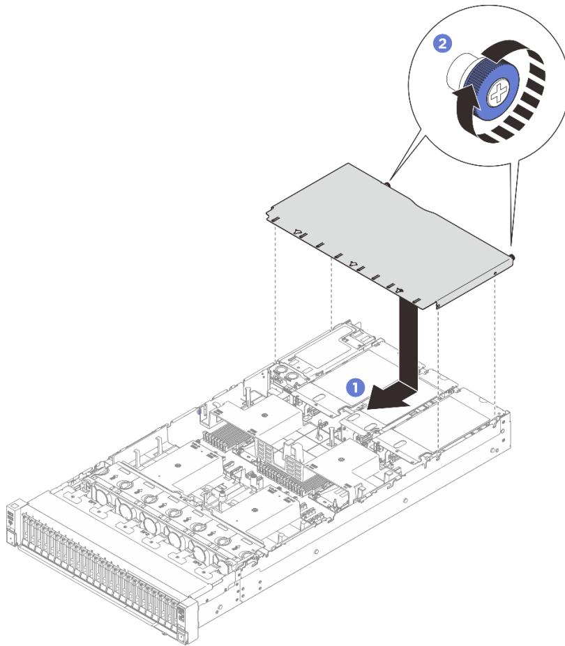
그림 235. 뒤쪽 윗면 덮개 설치
