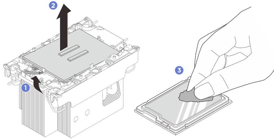
그림 193. 방열판 및 캐리어에서 프로세서 분리 중
