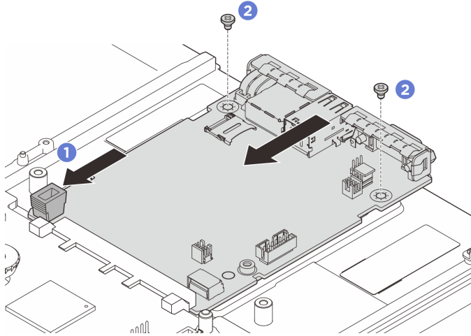
그림 226. 시스템 I/O 보드 설치
