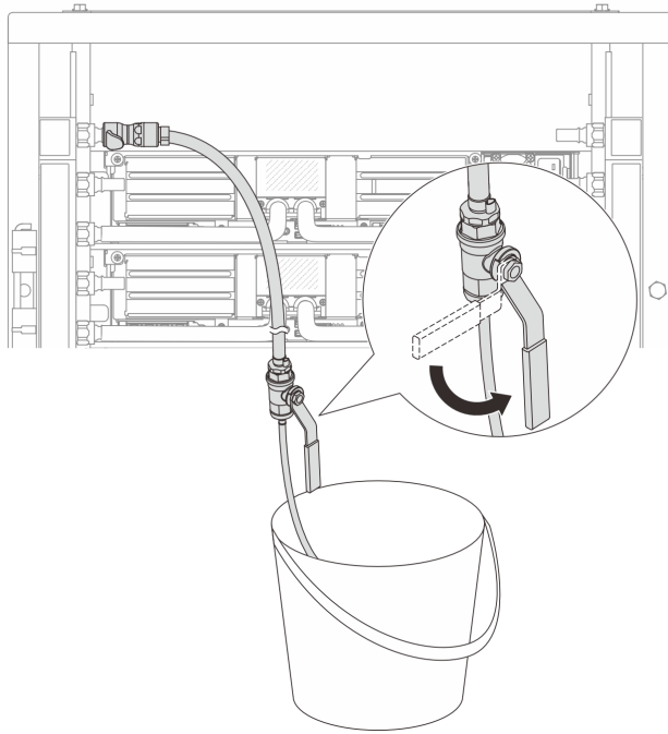
그림 150. 공급 측 블리드 밸브 열기
