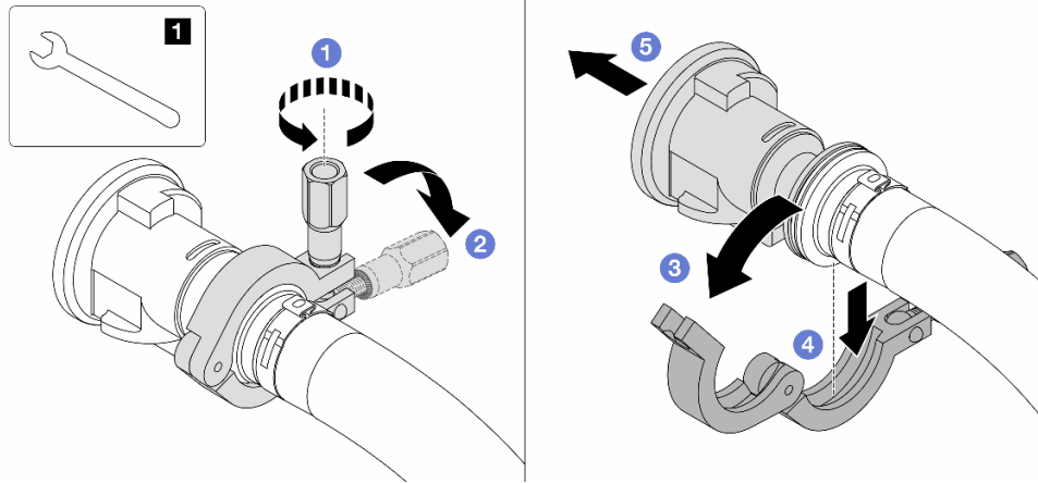
그림 120. 볼 밸브 분리
