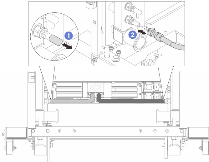
그림 126. 퀵 커넥트 플러그 설치
