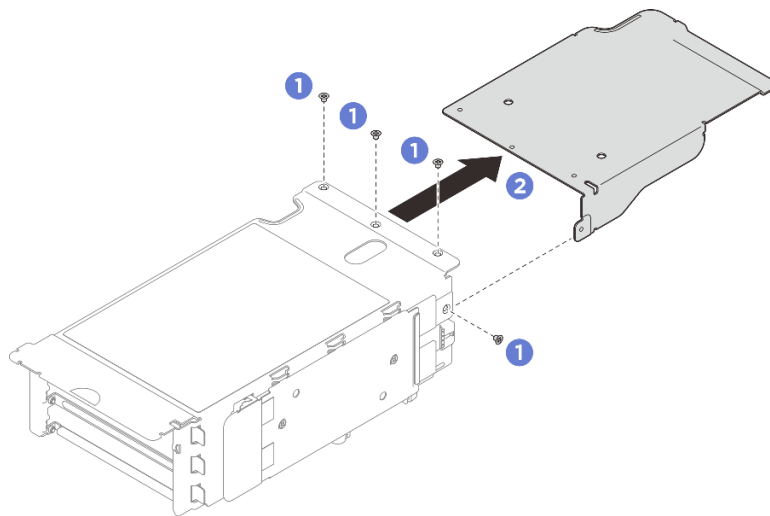
그림 183. PCIe 라이저 확장기 제거
