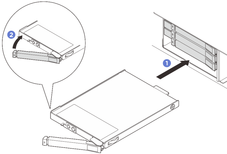
그림 41. E3.S 핫 스왑 드라이브 설치
