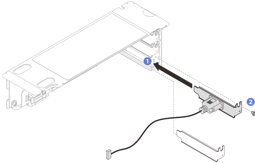
그림 219. 직렬 포트 모듈 설치
