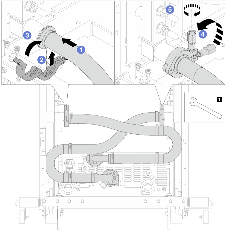
그림 122. 연결 세트 설치
