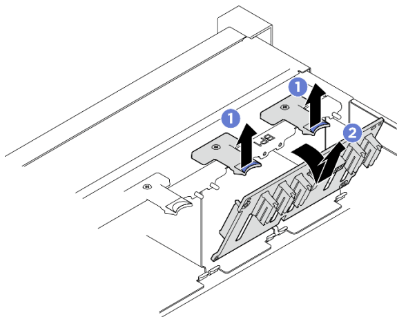
그림 5. 2.5인치 드라이브 백플레인 제거
