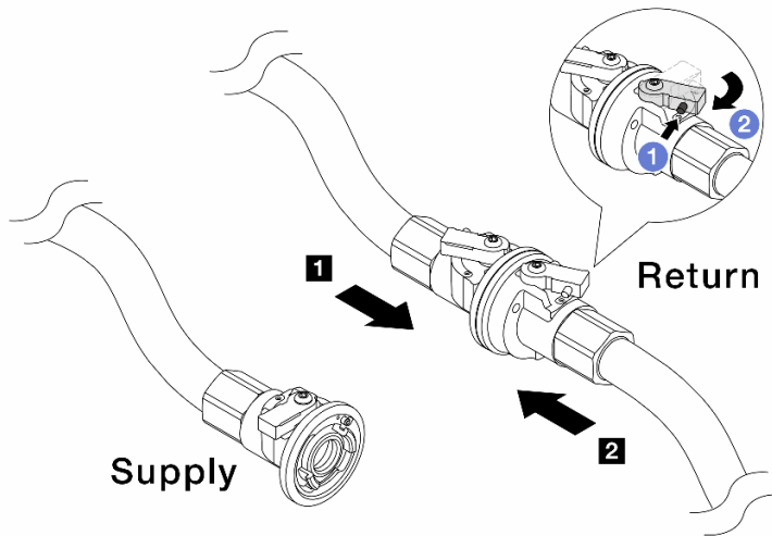
그림 145. 매니폴드 리턴에 설비 공급
