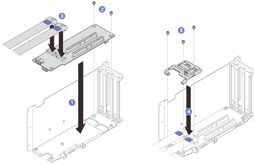
그림 178. PCIe 라이저 카드 설치
