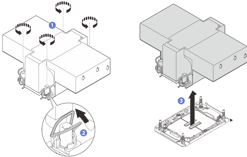
그림 192. 2U 성능 PHM 제거
