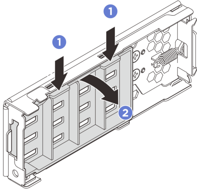
그림 43. 내부 플레이트 제거
