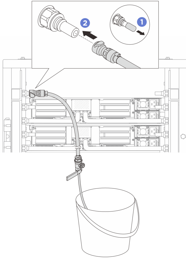
그림 127. 공급 측에 블리드 키트 설치
