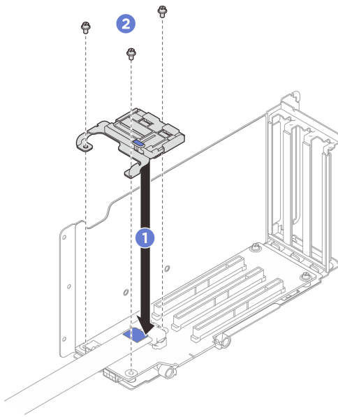
그림 182. PCIe 고정장치 설치
