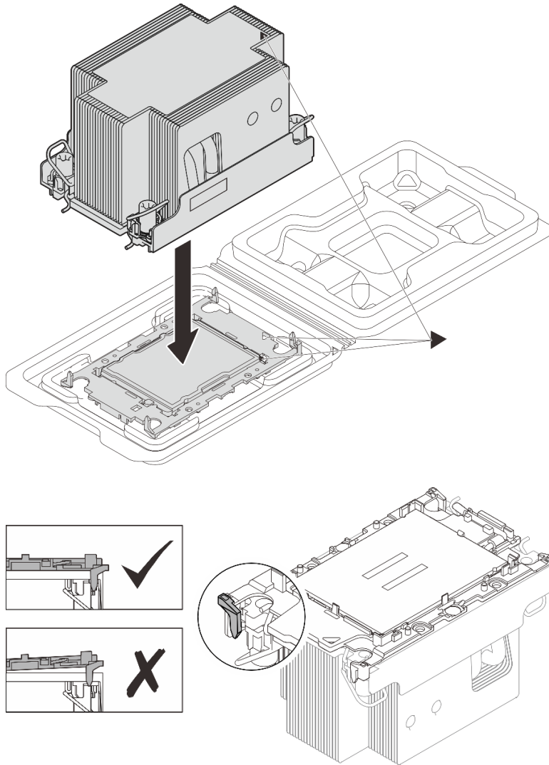
그림 198. 운송 트레이 내 프로세서로 PHM 조립
