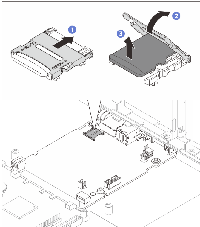
그림 156. MicroSD 카드 제거
