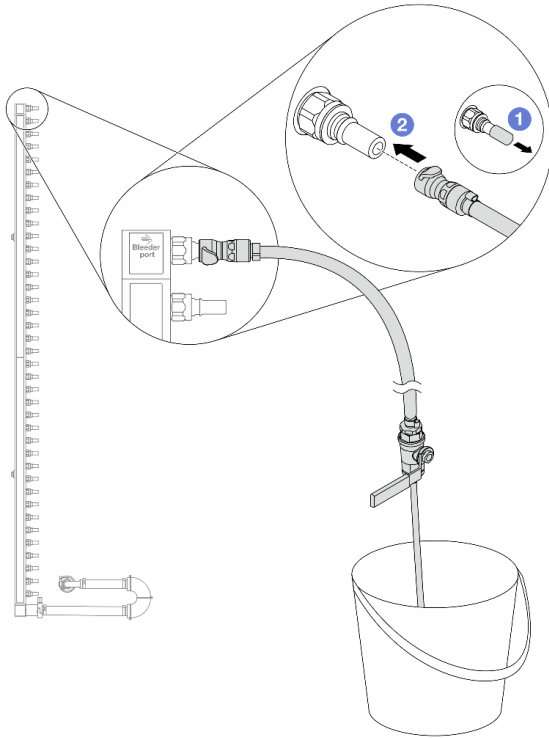
그림 114. 공급 측에 블리드 키트 설치
