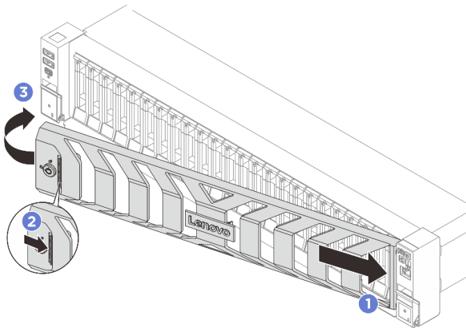
그림 216. 보안 베젤 설치
