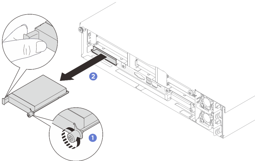
그림 158. OCP 모듈 제거
