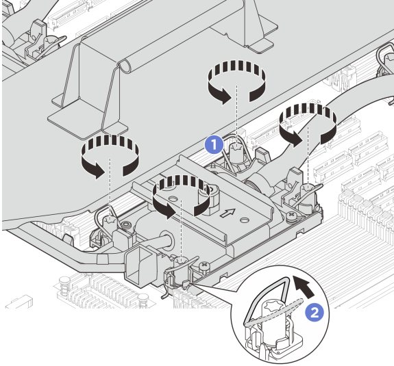
그림 82. Torx T30 너트 풀기
