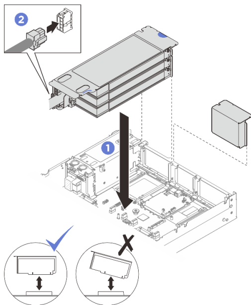
그림 171. PCIe LP 라이저 설치(전원 커넥터 포함)
