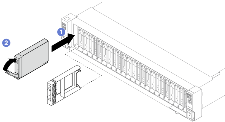
그림 7. 2.5인치 핫 스왑 드라이브 설치
