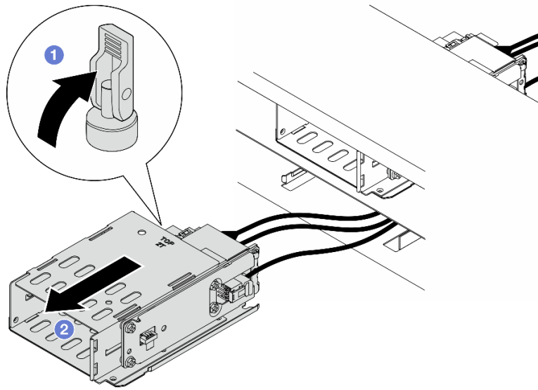
그림 33. E3.S 2T 케이스 제거
