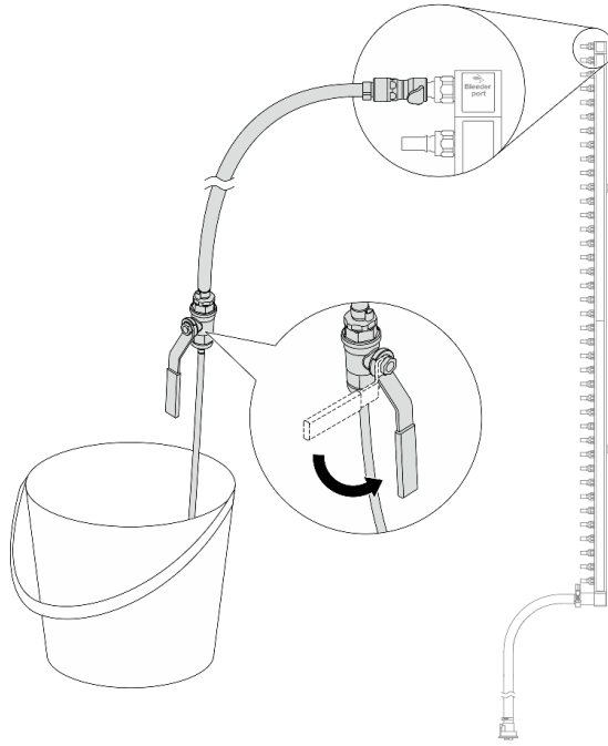
그림 139. 블리드 밸브 열기
