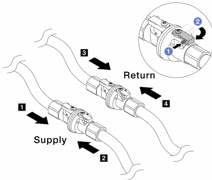
그림 151. 볼 밸브 열기
