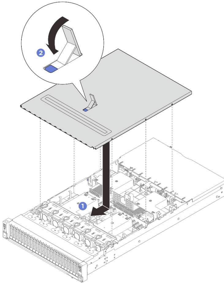
그림 236. 앞쪽 윗면 덮개 설치
