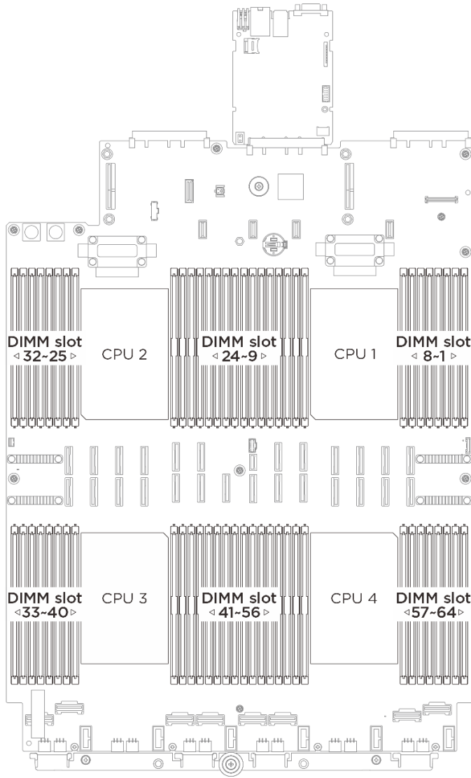
그림 154. 메모리 모듈 및 프로세서 레이아웃
