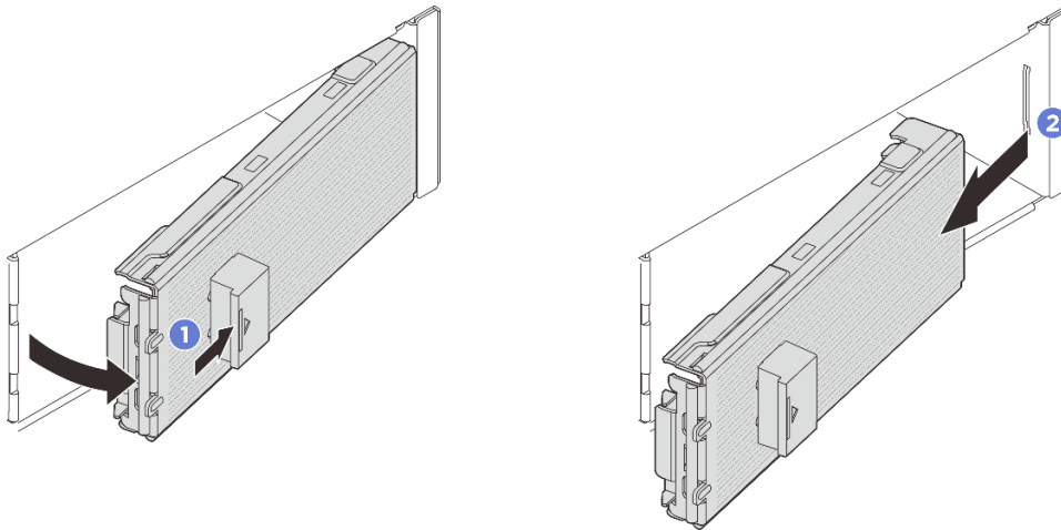
그림 24. E3.S 베젤 제거
