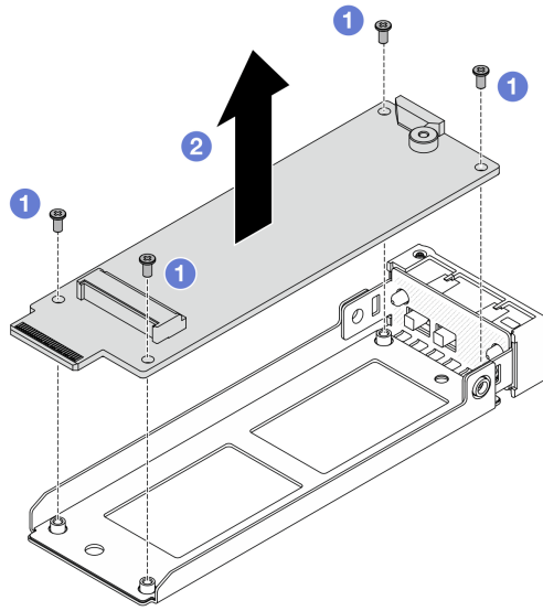
그림 66. M.2 인터포저 제거
