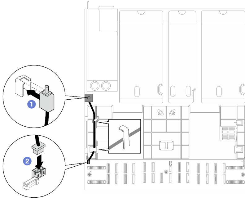
그림 76. 침입 스위치 설치
