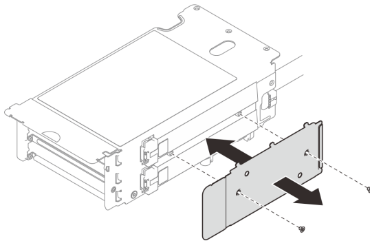
그림 174. 케이블 덮개 제거
