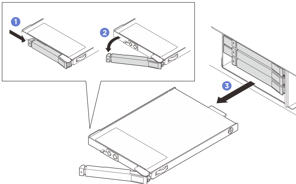
그림 38. E3.S 핫 스왑 드라이브 제거
