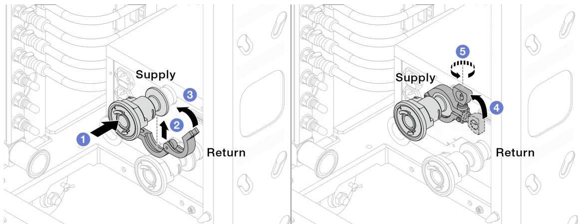
그림 121. 볼 밸브 설치
