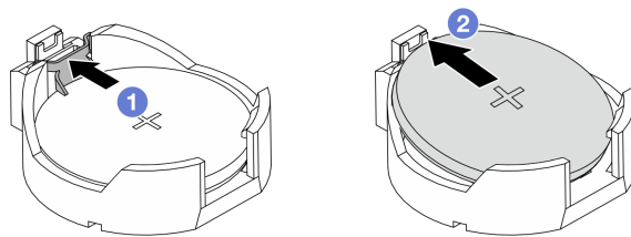
그림 21. CMOS 배터리 제거
