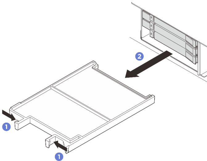
그림 40. 베이 필터 제거
