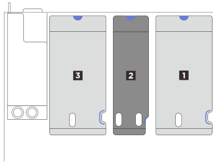
그림 168. PCIe 라이저 3개가 지원되는 서버 모델
