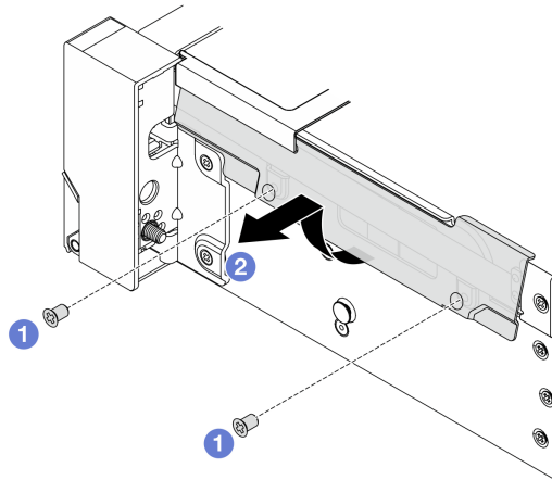
그림 201. 케이블 고정장치 제거
