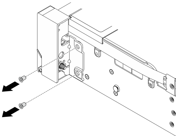
그림 202. 나사 제거
