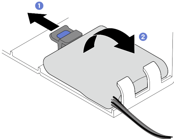
그림 54. 플래시 전원 모듈 제거
