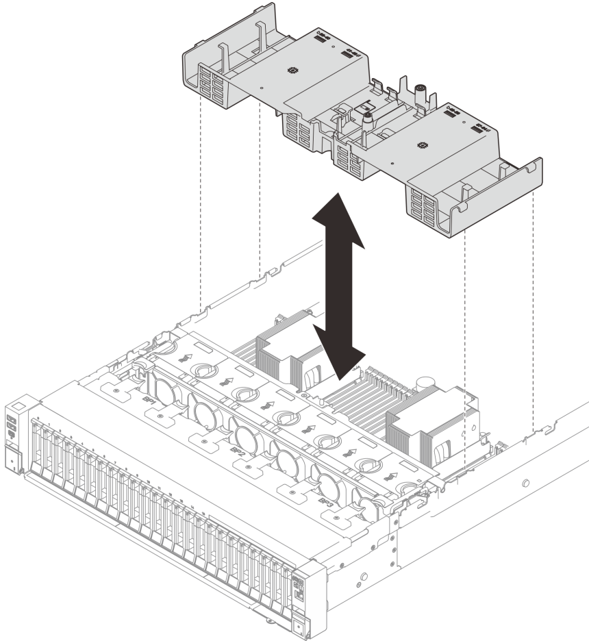
그림 11. 앞면 공기 조절 장치 설치
