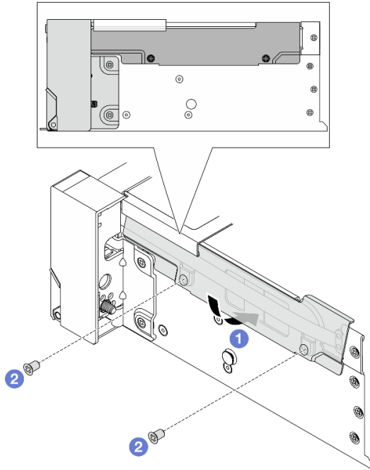
그림 206. 케이블 고정장치 설치
