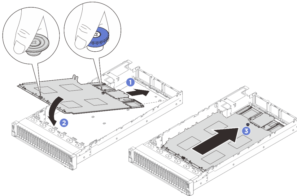
그림 231. 시스템 보드 어셈블리 설치
