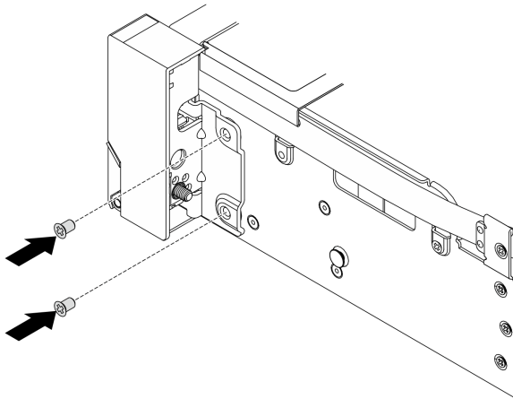
그림 205. 나사 설치
