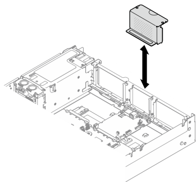
그림 78. 라이저 필러 제거
