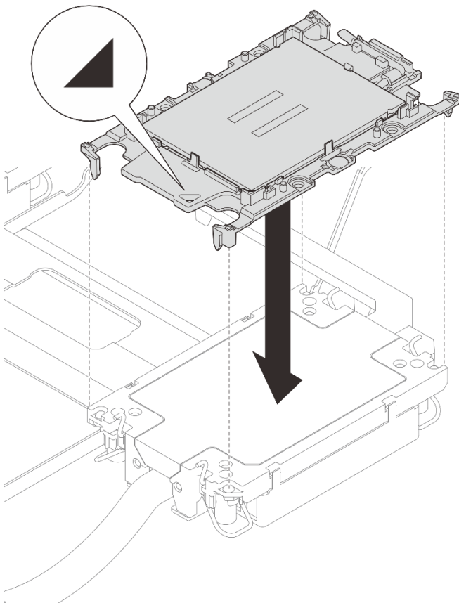
그림 87. 냉각판에 프로세서 설치
