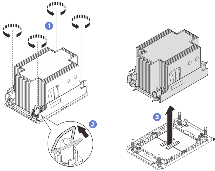
그림 191. 2U 표준 PHM 제거
