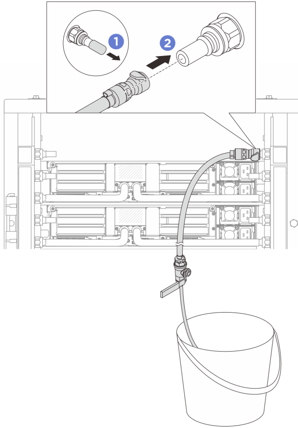
그림 147. 리턴 측에 블리드 키트 설치
