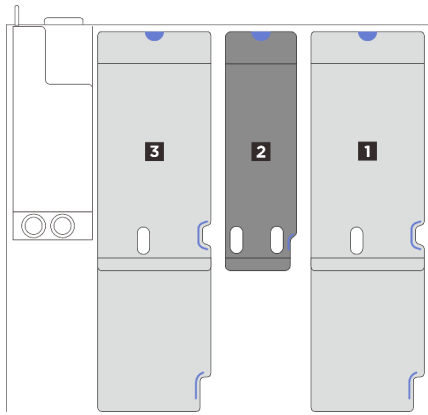
그림 161. PCIe 라이저 3개 및 라이저 확장기가 있는 서버 모델
