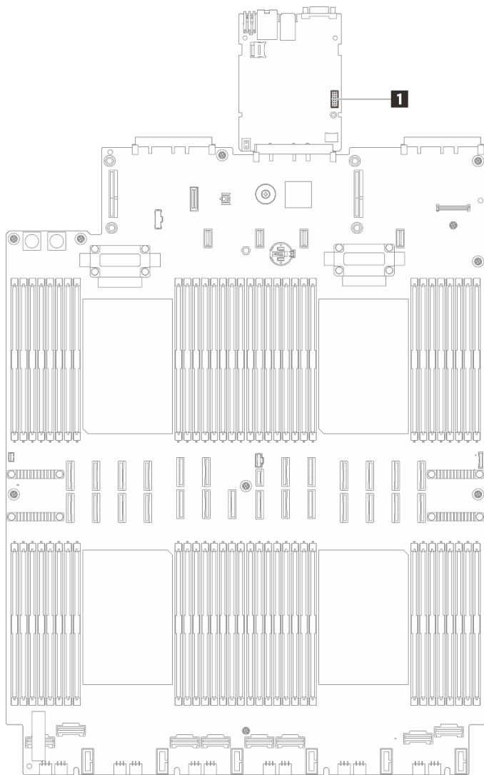
그림 220. 직렬 포트 커넥터 위치
