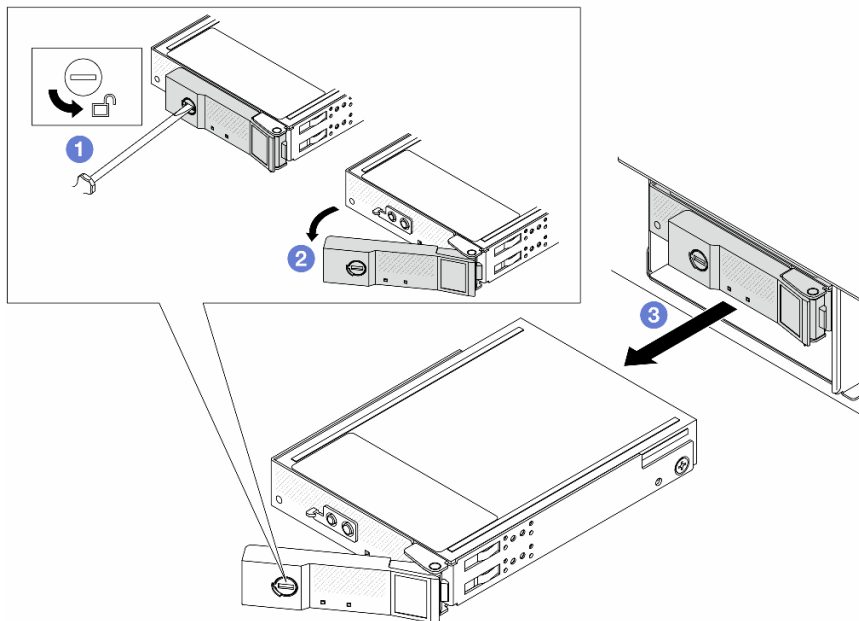
그림 25. CMM 제거
