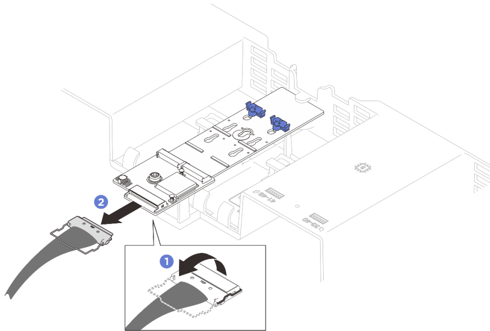
그림 9. M.2 부트 어댑터 케이블 분리
