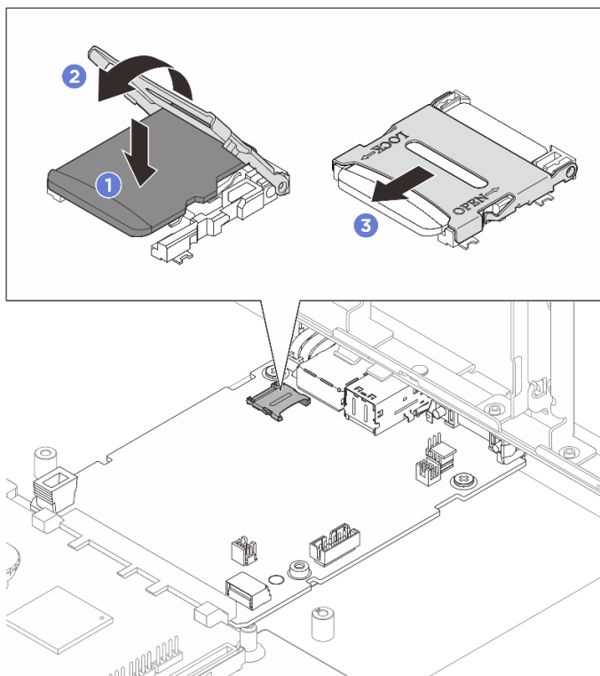
그림 157. microSD 카드 설치
