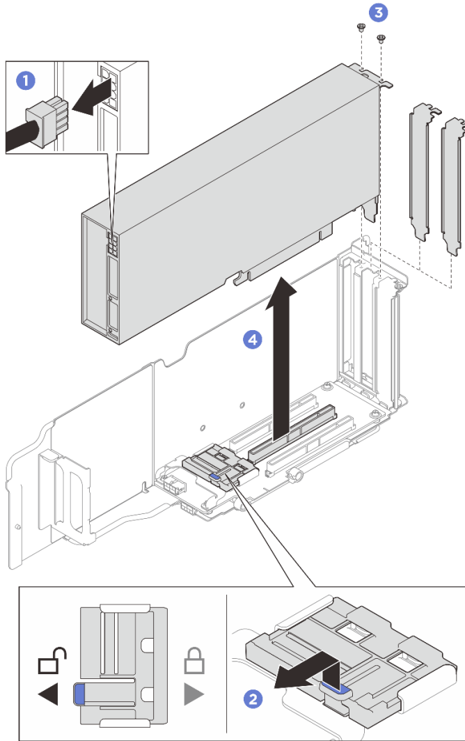
그림 59. 더블 와이드 GPU 어댑터 제거
