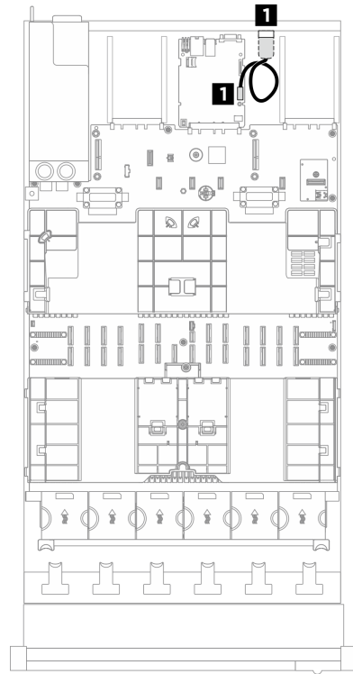
그림 222. PCIe 라이저 4개가 지원되는 서버 모델의 직렬 포트 모듈 케이블 배선
