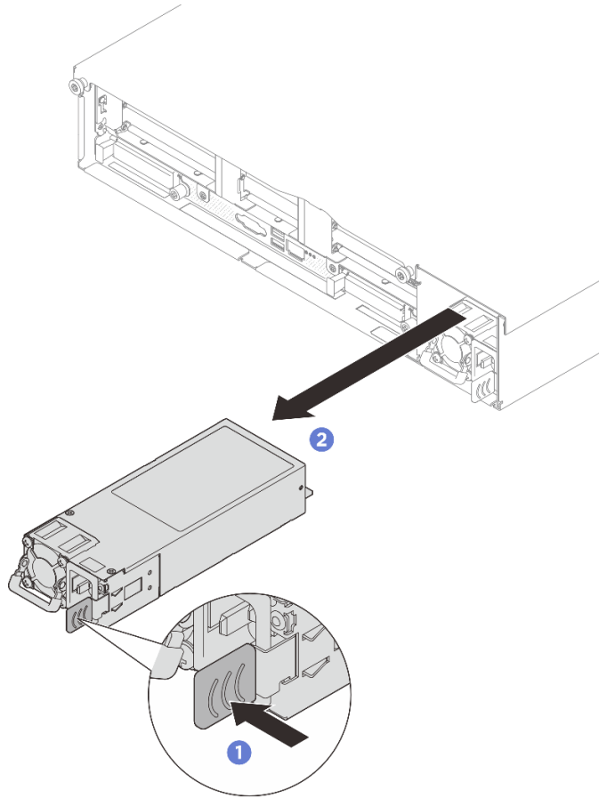
그림 188. 전원 공급 장치 제거
