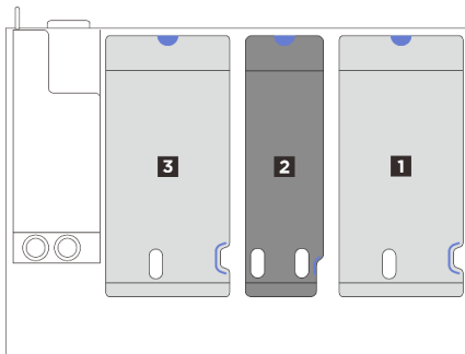
그림 160. PCIe 라이저 3개가 지원되는 서버 모델
