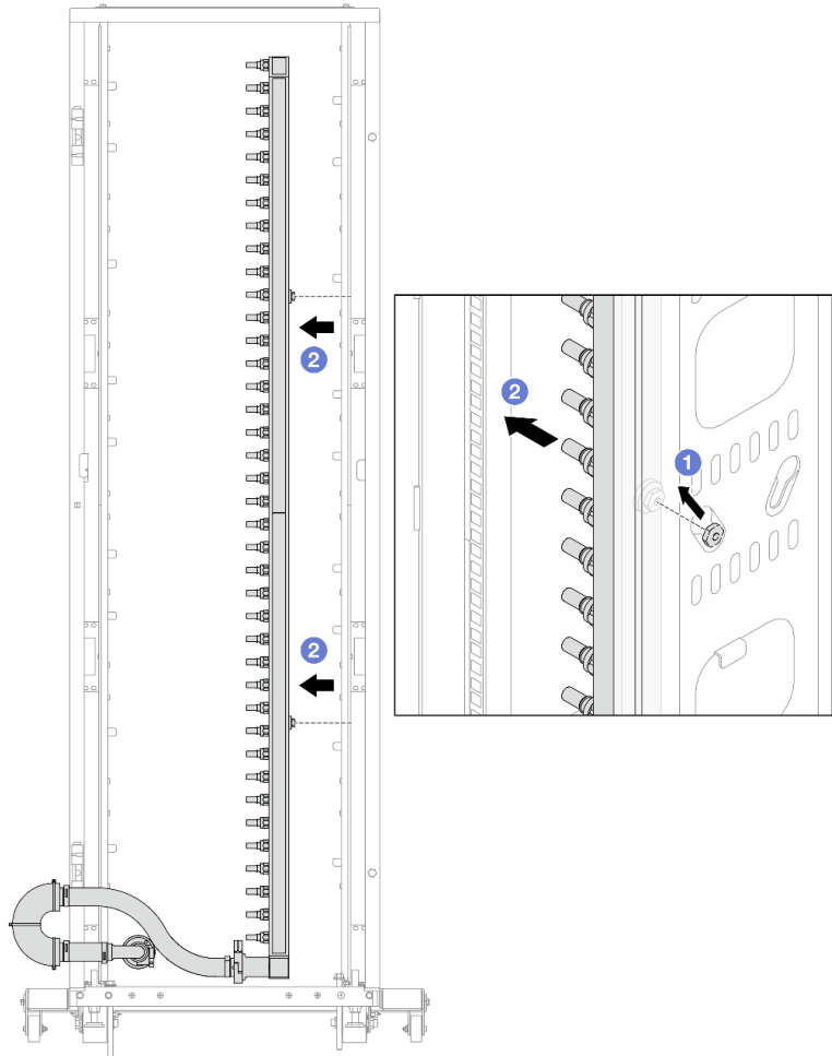
그림 113. 매니폴드 제거
