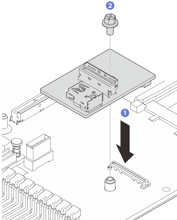
그림 239. USB I/O 보드 설치
