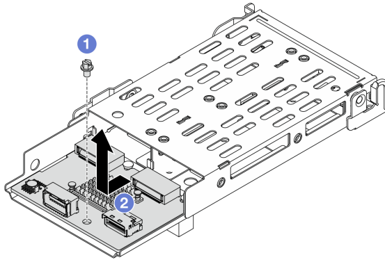
그림 208. M.2 부트 어댑터 제거
