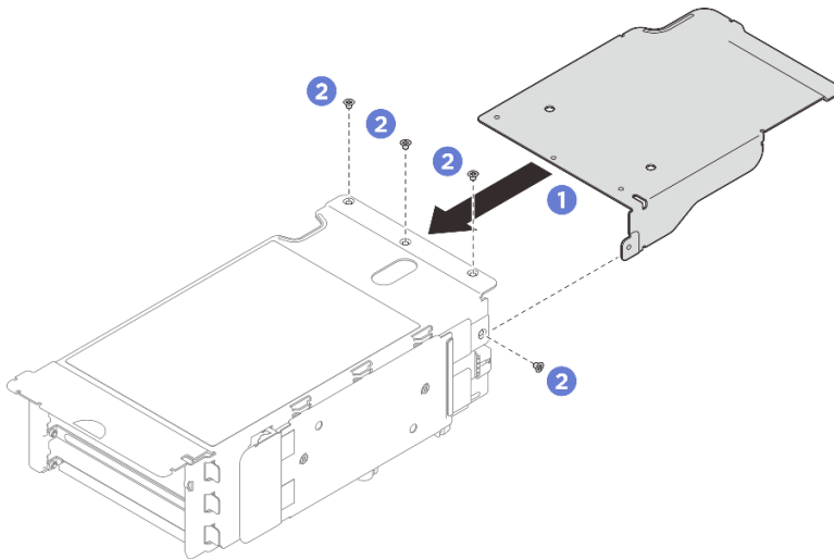
그림 184. PCIe 라이저 확장기 설치
