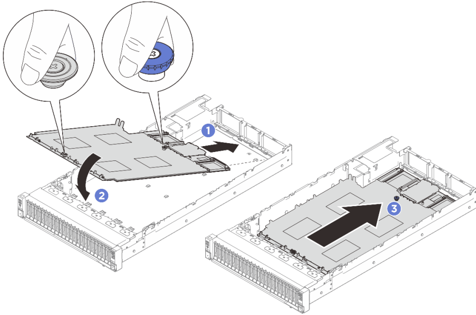
그림 227. 시스템 보드 어셈블리 설치
