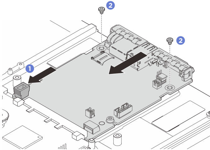
그림 230. 시스템 I/O 보드 설치
