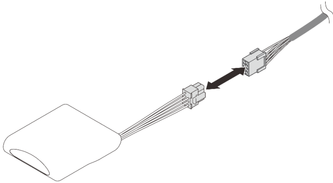
그림 53. 플래시 전원 모듈 케이블 분리
