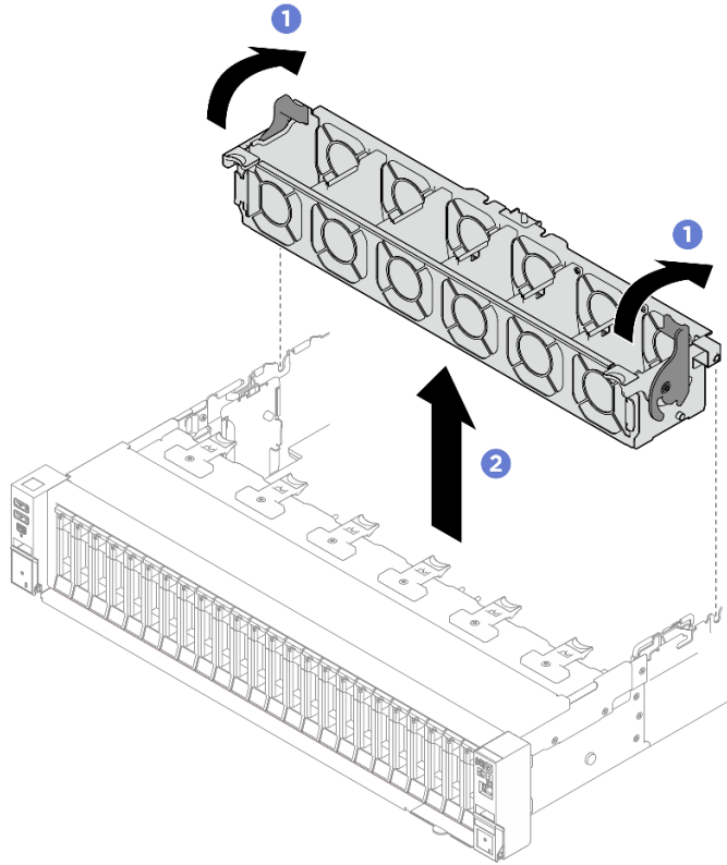
그림 50. 팬 케이지 제거
