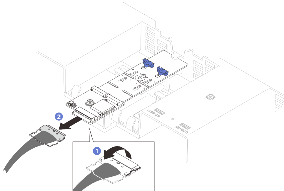
그림 97. M.2 부트 어댑터 케이블 분리
