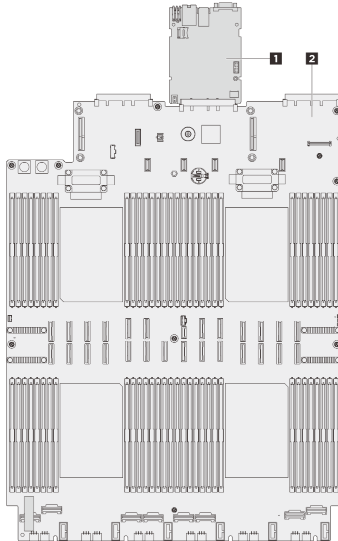
그림 223. 시스템 보드 어셈블리 레이아웃
