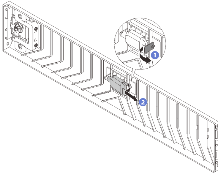
그림 215. 키 제거
