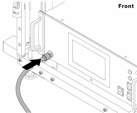
그림 124. CDU 앞면
