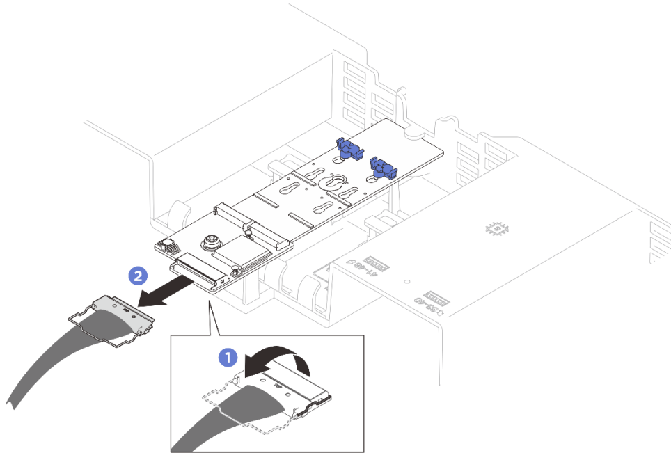
그림 15. M.2 부트 어댑터 케이블 분리
