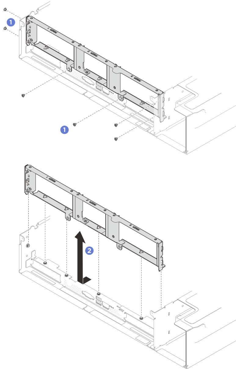
그림 211. 뒷면 벽 제거
