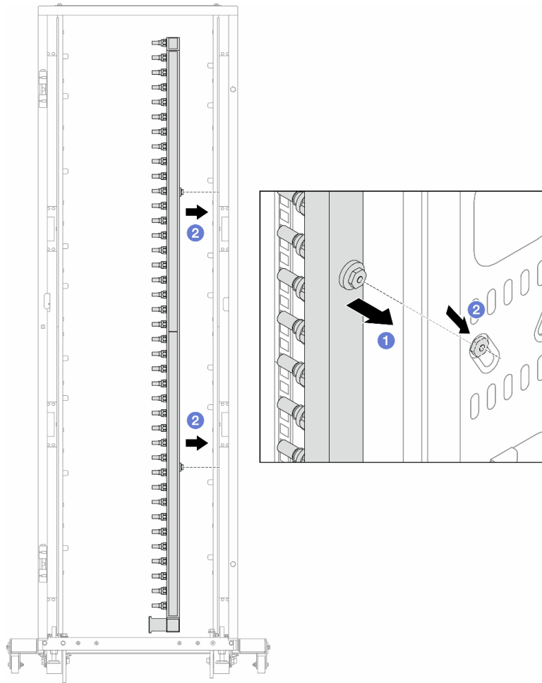
그림 119. 매니폴드 설치
