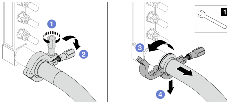
그림 140. 호스 키트에서 매니폴드 분리
