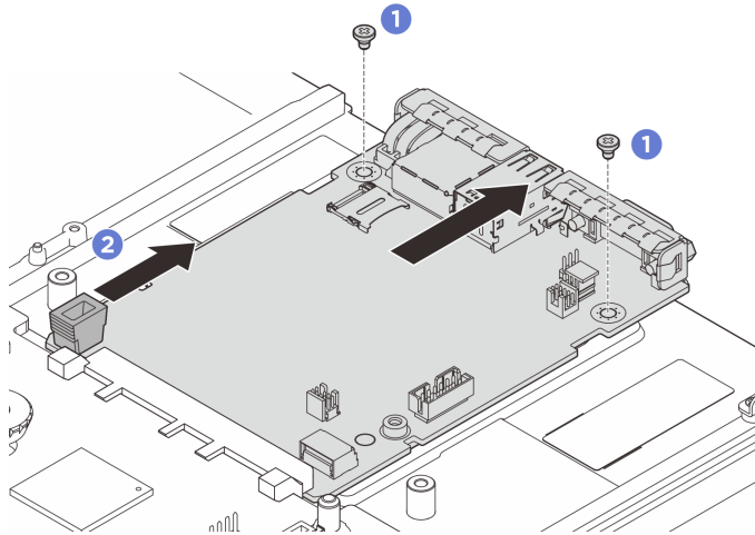
그림 225. 시스템 I/O 보드 제거
