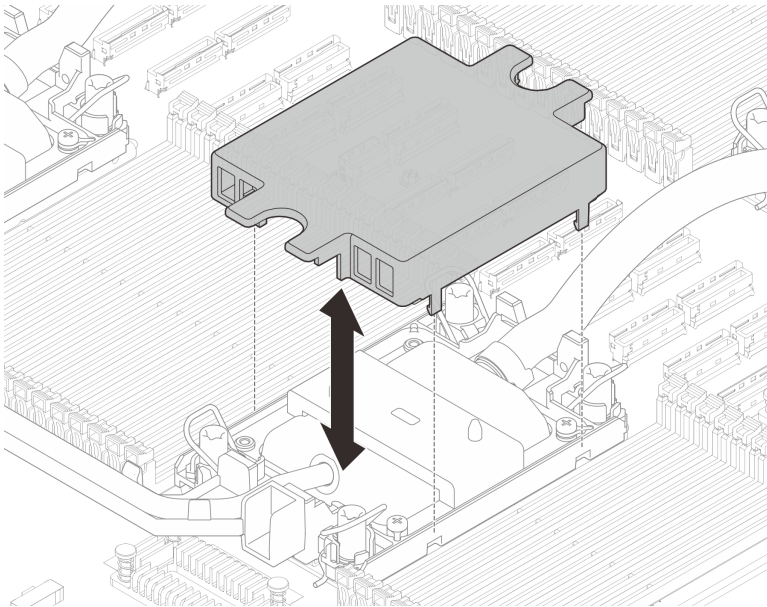
그림 93. 냉각판 덮개 설치
