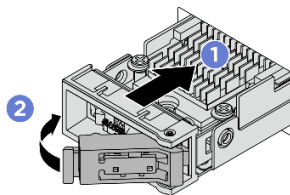
그림 74. M.2 드라이브 어셈블리 설치
