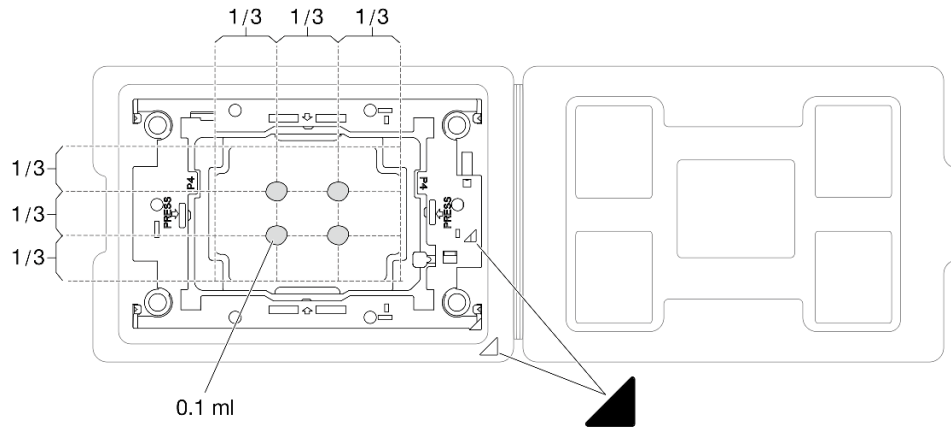
그림 86. 운송 트레이 내 프로세서에 열전도 그리스 도포
