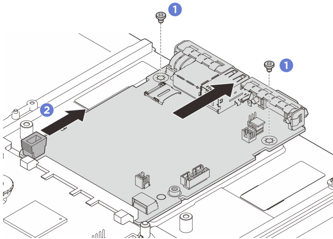
그림 229. 시스템 I/O 보드 제거
