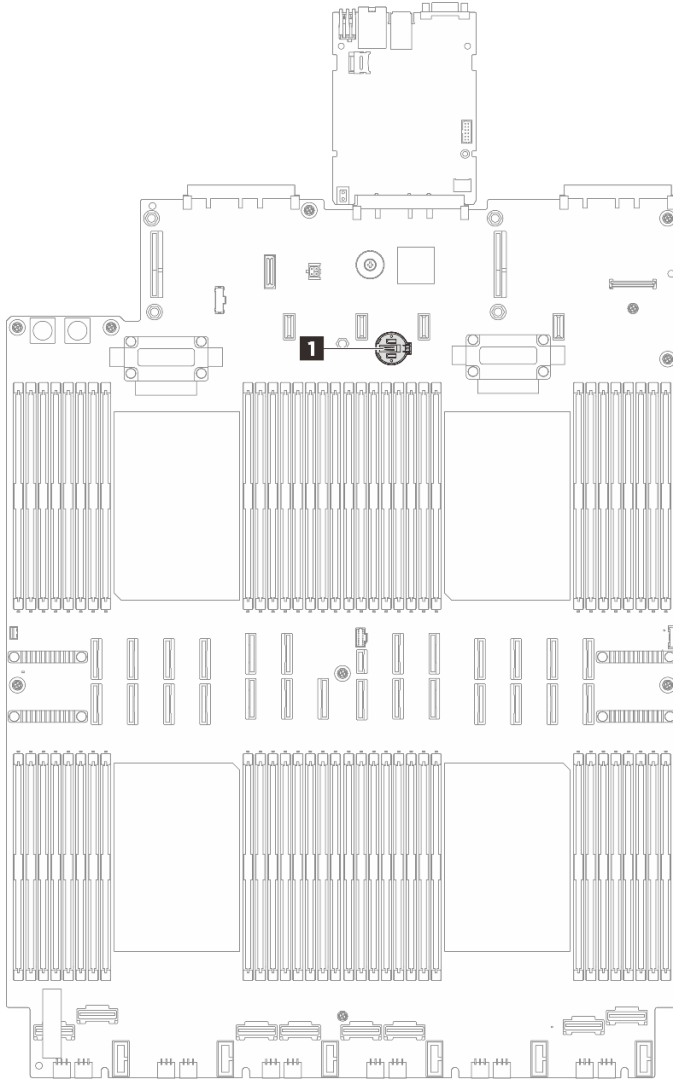
그림 20. CMOS 배터리 위치
