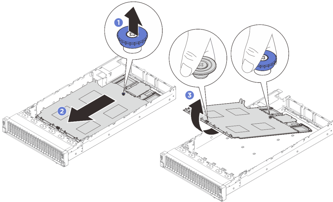
그림 224. 시스템 보드 어셈블리 제거
