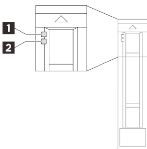
그림 243. 2.5인치 드라이브 LED
