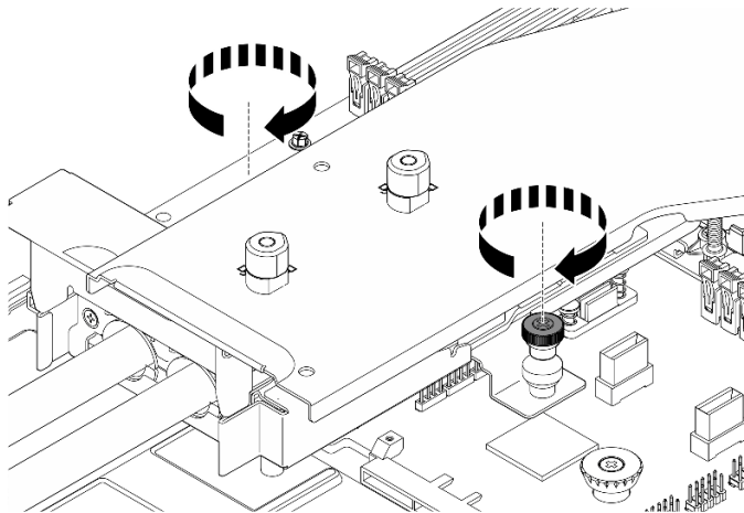
그림 89. 냉각판 어셈블리 설치
