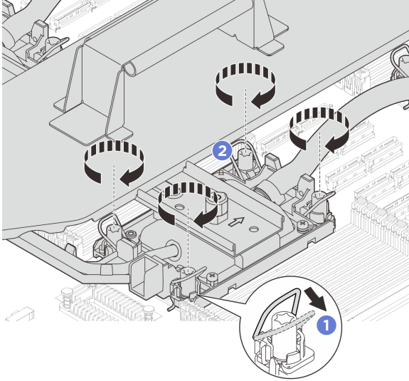
그림 90. Torx T30 너트 조이기
