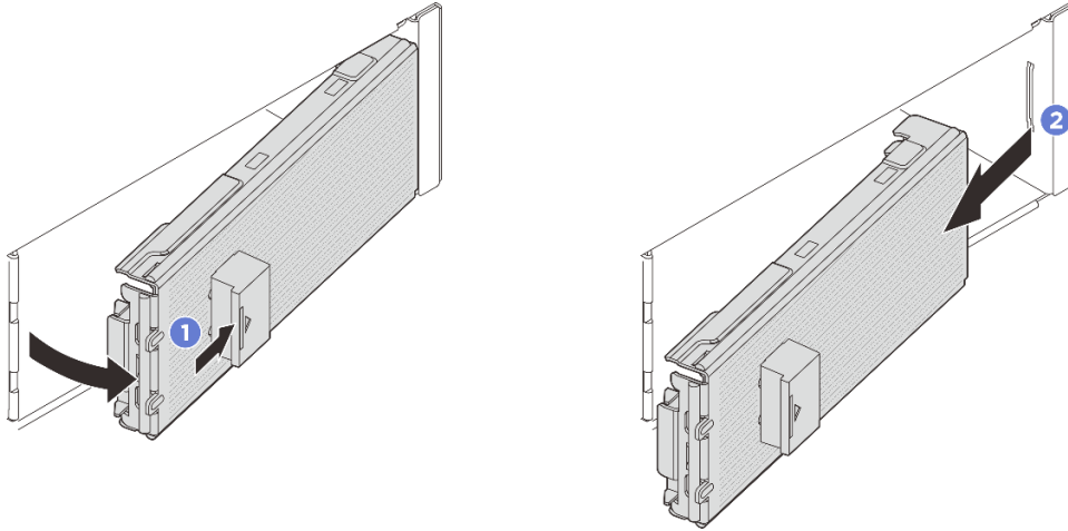
그림 37. E3.S 베젤 제거
