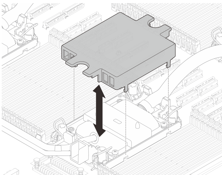
그림 79. 냉각판 덮개 제거
