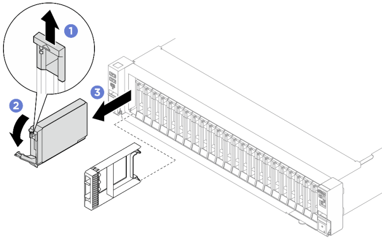
그림 4. 2.5인치 핫 스왑 드라이브 제거
