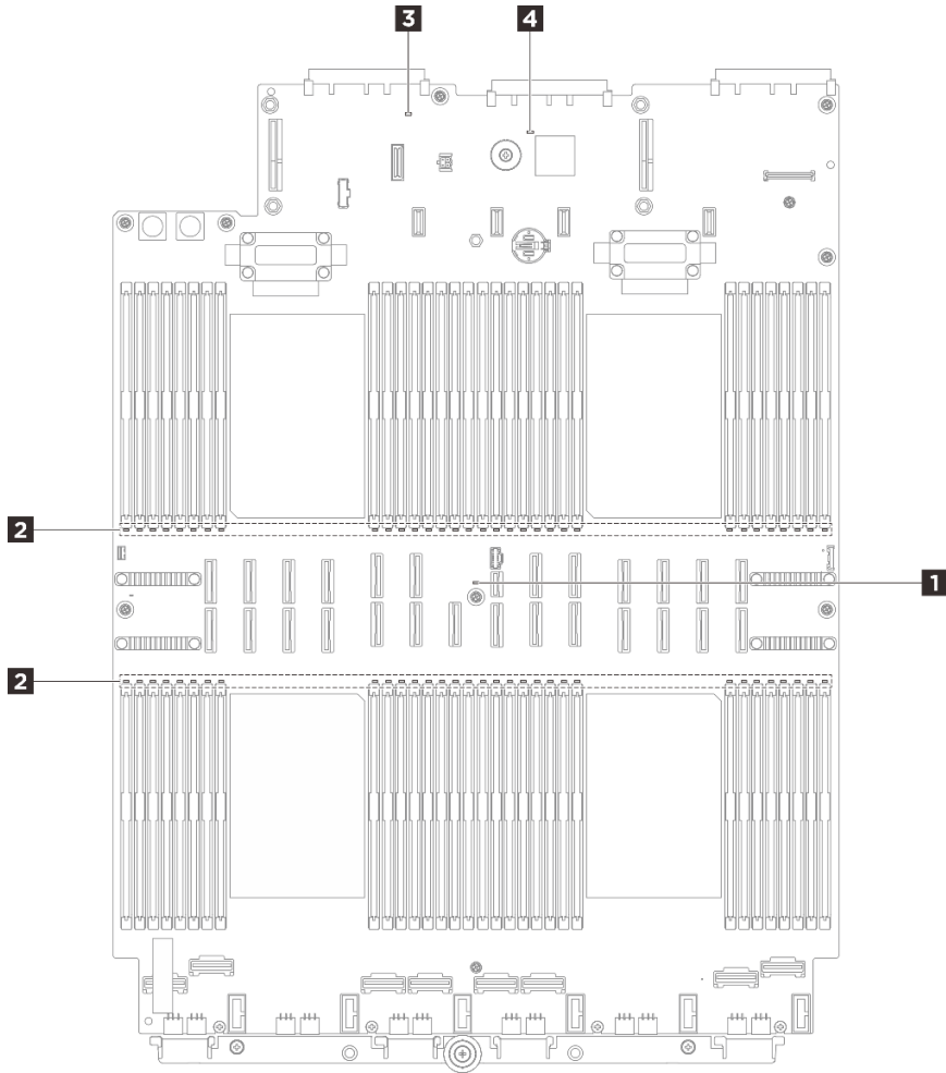
그림 254. 프로세서 보드 LED
