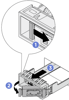
그림 73. M.2 드라이브 트레이 제거
