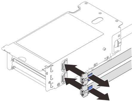
그림 179. 케이블 연결
