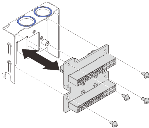
그림 186. 전원 분배 보드 분리
