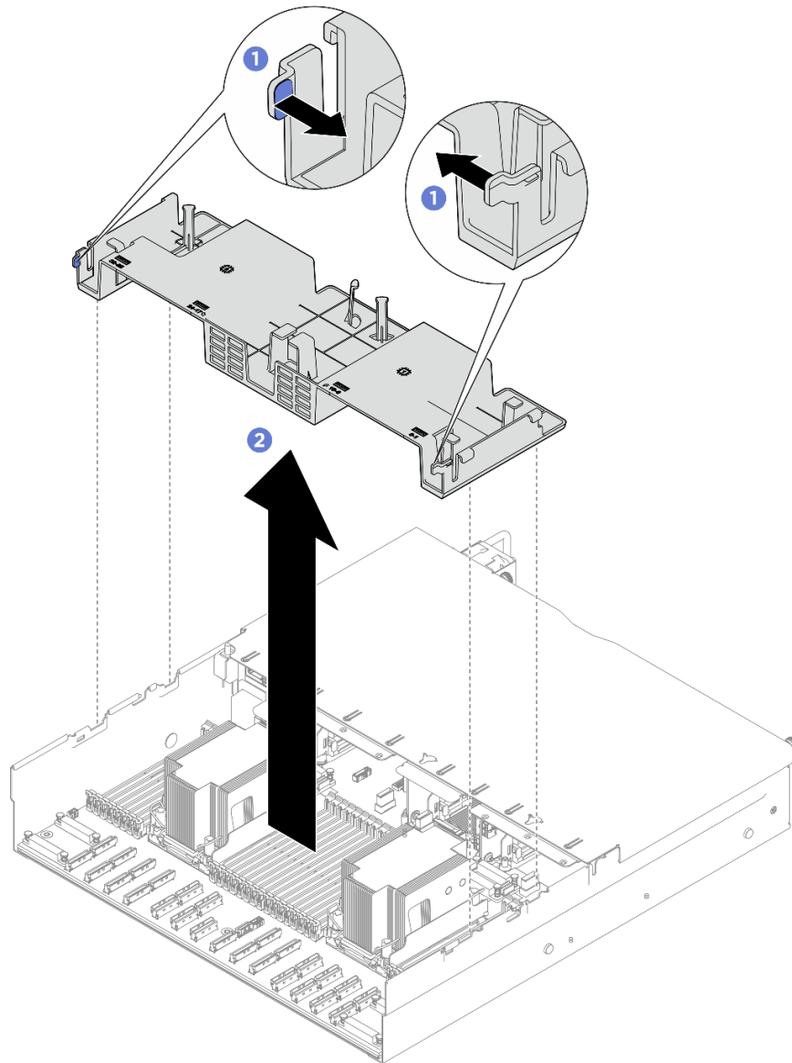
그림 16. 뒷면 공기 조절 장치 제거
