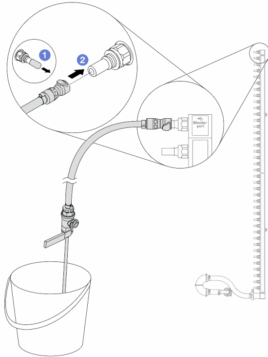
그림 116. 리턴 측에 블리드 키트 설치
