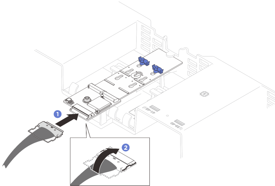
그림 18. M.2 부트 어댑터 케이블 연결
