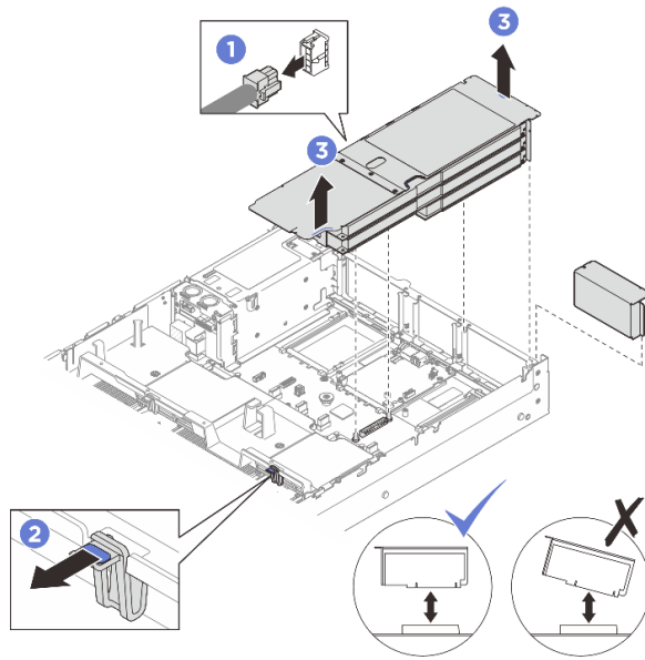
그림 165. PCIe FHFL 라이저 제거
