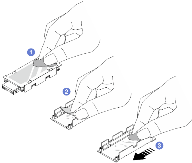
그림 68. 방열판 및 바닥판 청소
