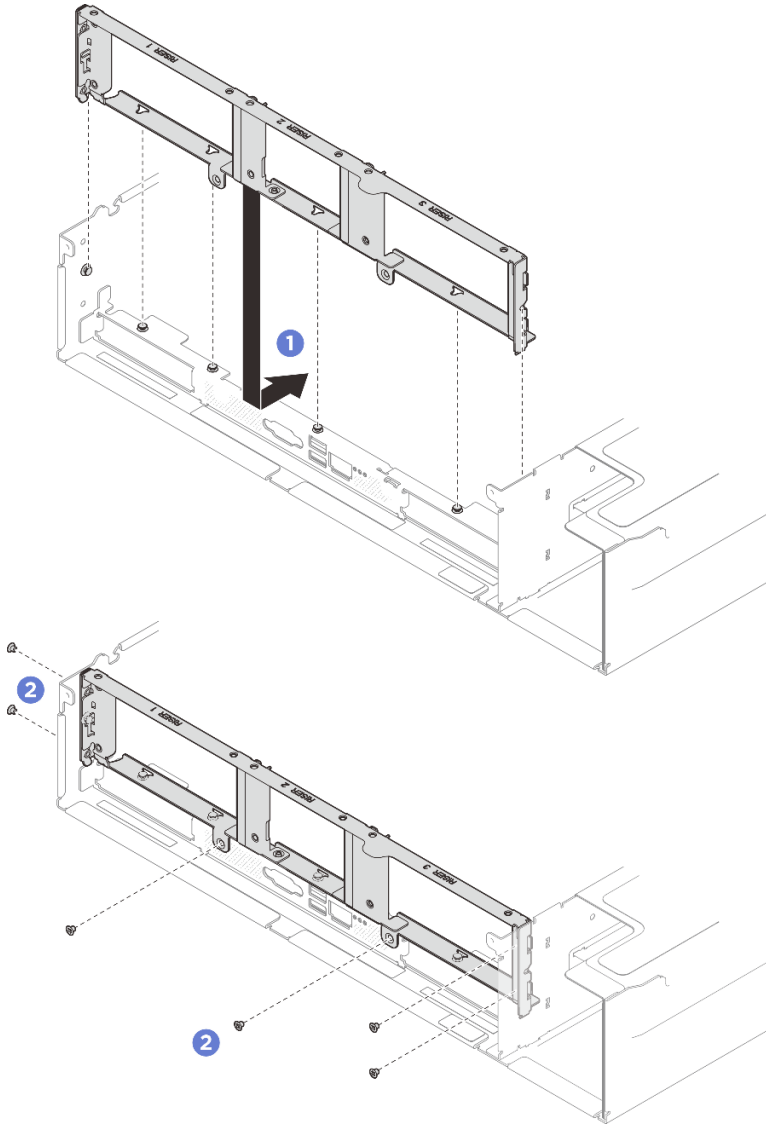
그림 212. 뒷면 벽 설치
