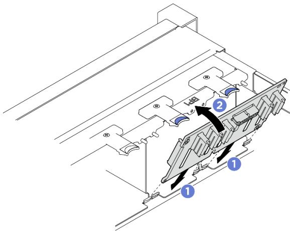
그림 6. 2.5인치 드라이브 백플레인 설치
