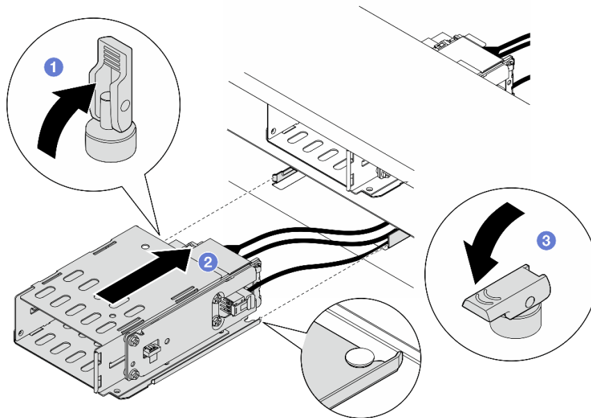
그림 36. E3.S 2T 케이스 설치
