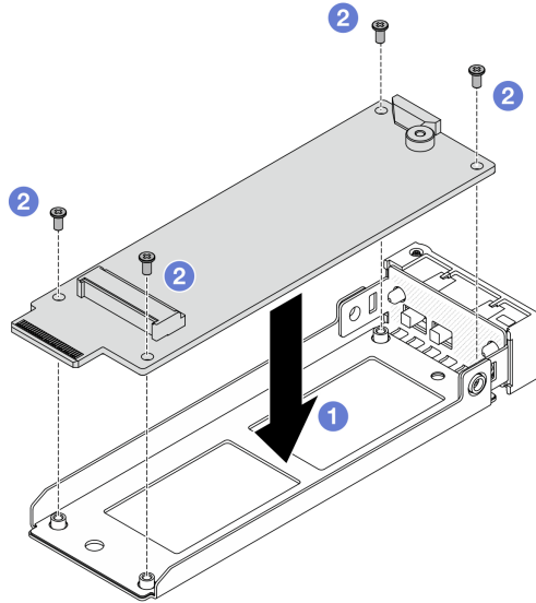
그림 71. M.2 인터포저 설치
