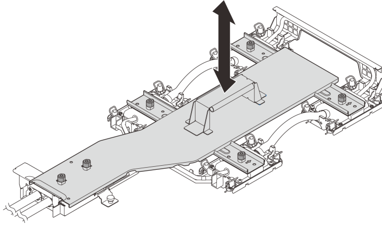
그림 80. 냉각판 캐리어 설치
