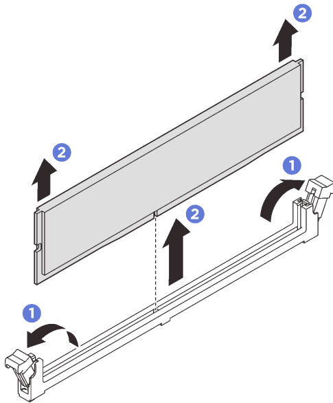
그림 153. 메모리 모듈 제거
