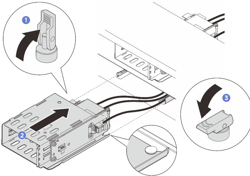
그림 48. E3.S 1T 케이스 설치
