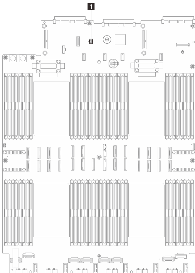
그림 95. 누수 감지 센서 모듈 연결
