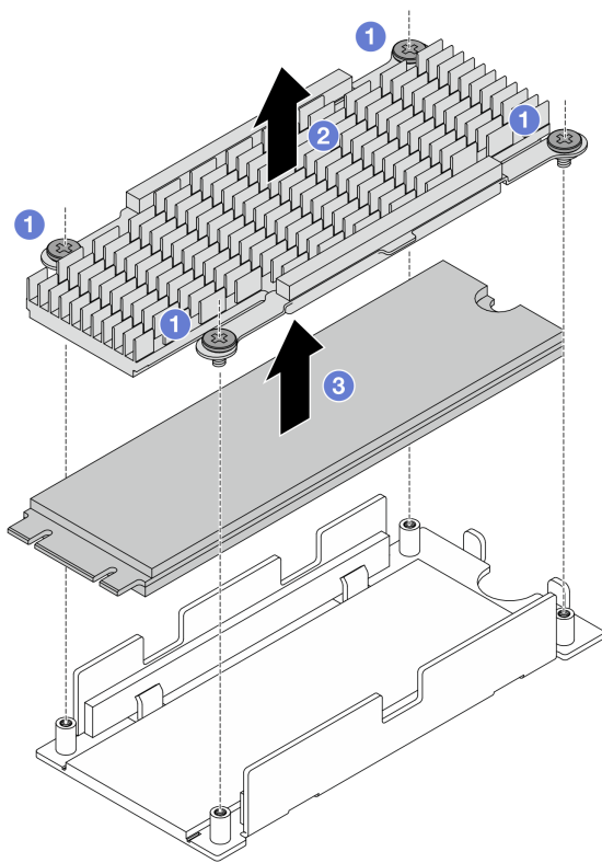
그림 67. M.2 드라이브 및 방열판 분리
