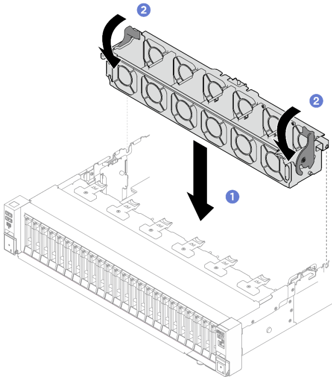
그림 51. 팬 케이스 설치
