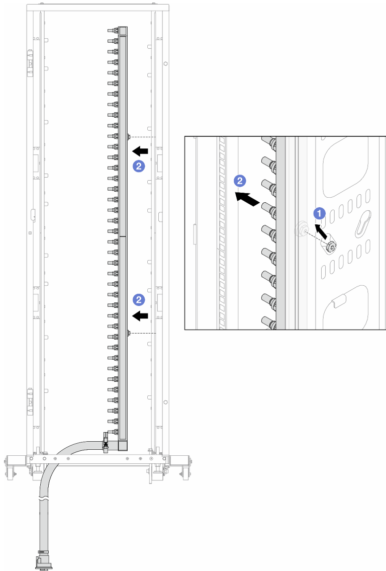
그림 135. 매니폴드 제거
