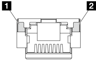
그림 256. XCC 시스템 관리 포트(10/100/1000Mbps RJ-45)의 LED
