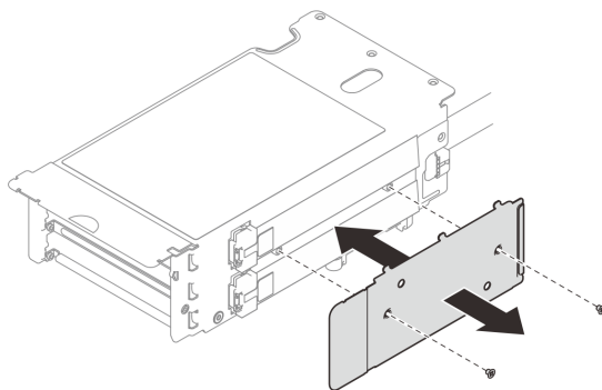
Рис. 174. Снятие кожуха кабелей
