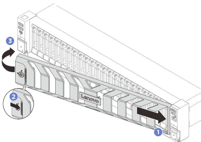
Рис. 216. Установка защитной панели
