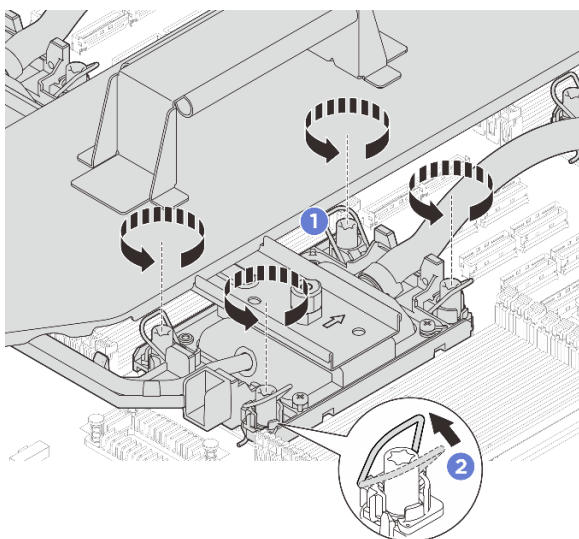
Рис. 82. Ослабление гаек Torx T30
