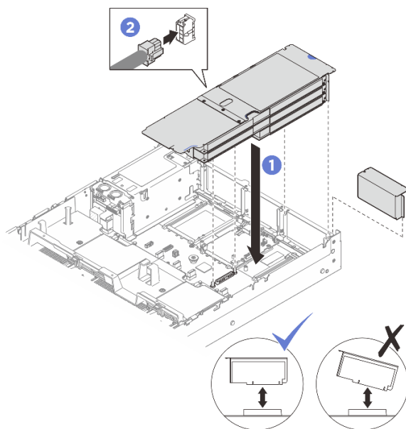
Рис. 173. Установка платы-адаптера Riser PCIe максимальной высоты, полной длины
