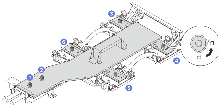
Рис. 91. Ослабление держателя платы охлаждения
