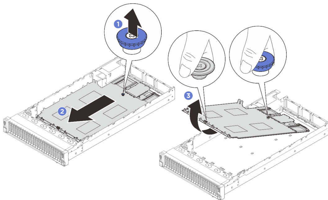
Рис. 228. Снятие блока материнской платы
