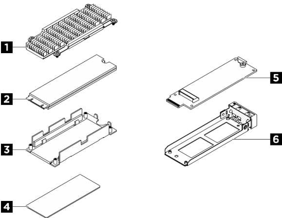
Рис. 62. Компоненты блока оперативно заменяемых дисков M.2
