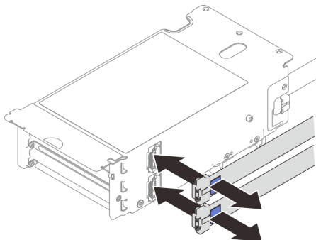
Рис. 179. Подключение кабелей
