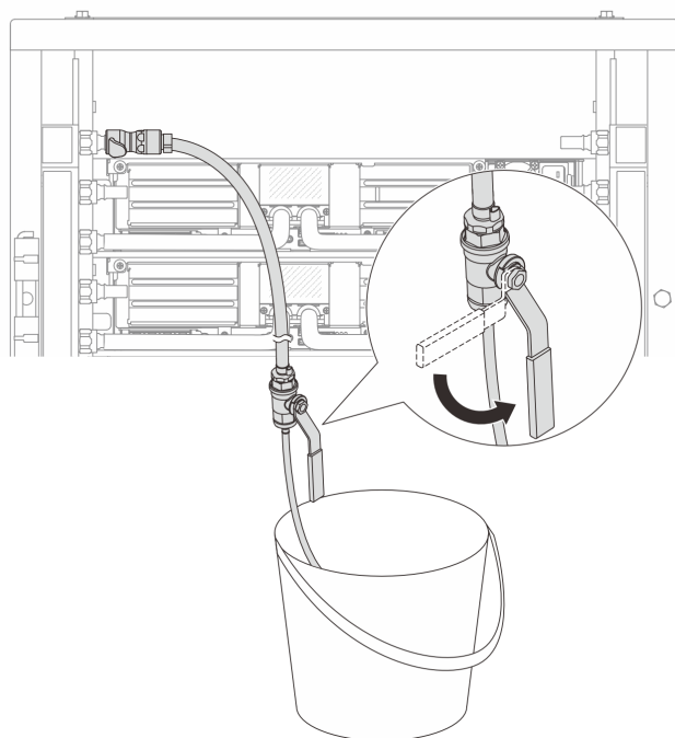
Рис. 146. Открытие клапана отводной трубки на стороне подачи
