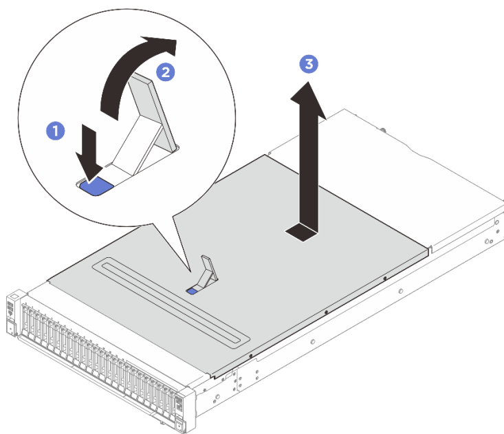
Рис. 233. Снятие переднего верхнего кожуха
