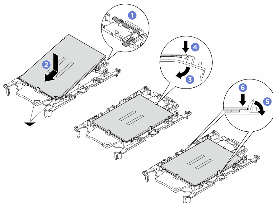
Рис. 85. Установка держателя процессора
