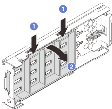
Рис. 31. Снятие внутренней пластины
