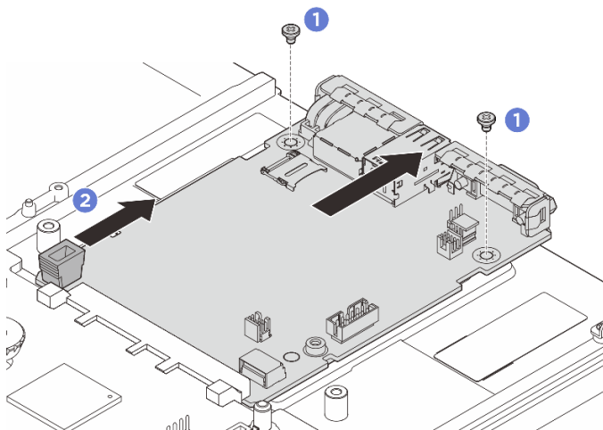
Рис. 229. Снятие системной платы ввода-вывода
