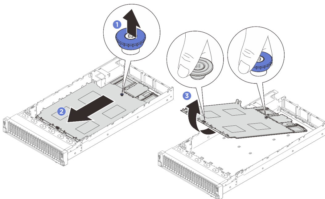
Рис. 224. Снятие блока материнской платы
