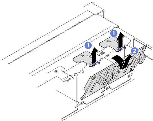
Рис. 5. Снятие объединительной панели для 2,5-дюймовых дисков
