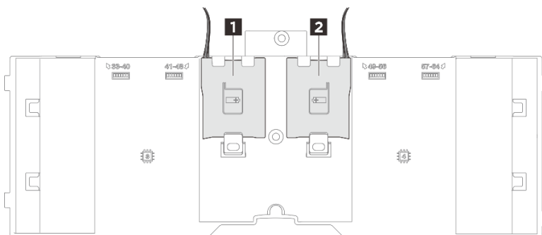
Рис. 55. Расположение гнезда модуля питания флэш-памяти
