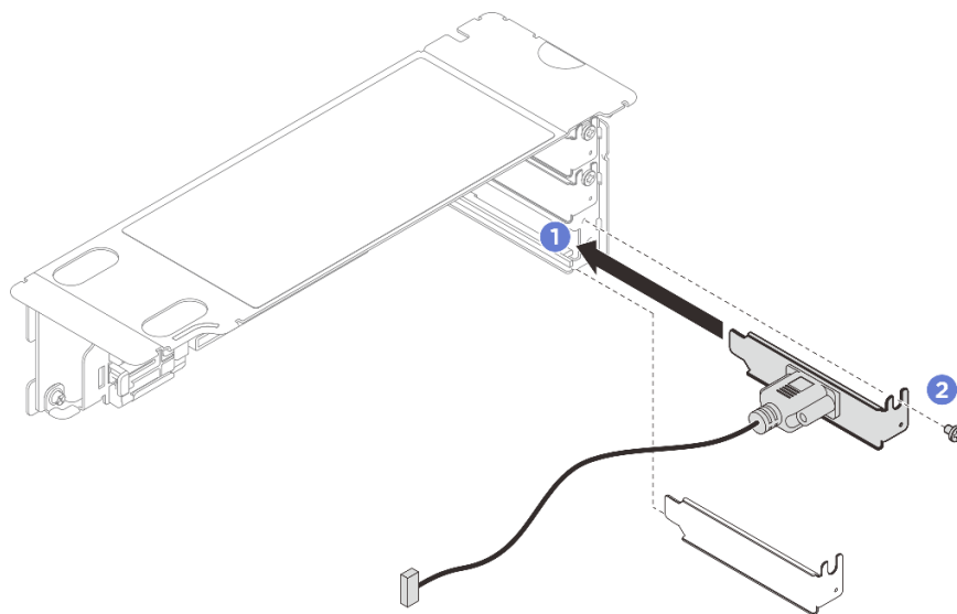
Рис. 219. Установка модуля последовательного порта
