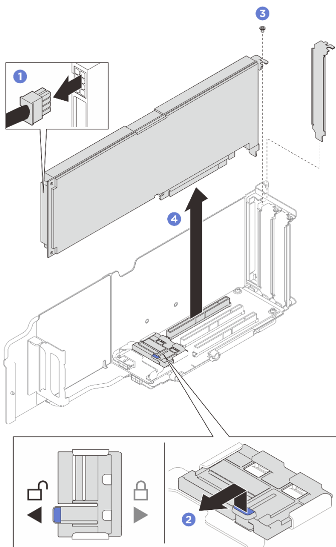
Рис. 58. Снятие адаптера графического процессора одинарной ширины
