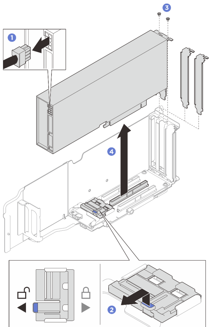
Рис. 59. Снятие адаптера графического процессора двойной ширины
