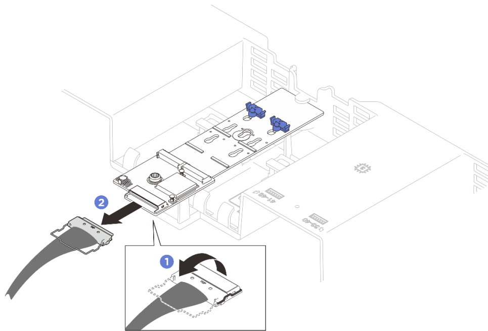
Рис. 9. Отключение кабеля адаптера загрузки M.2
