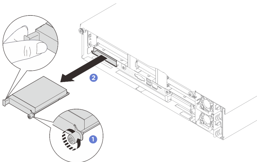
Рис. 158. Снятие модуля ОСР
