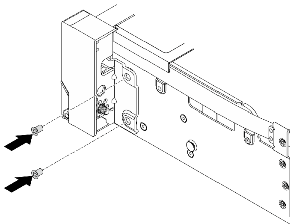
Рис. 205. Установка винтов
