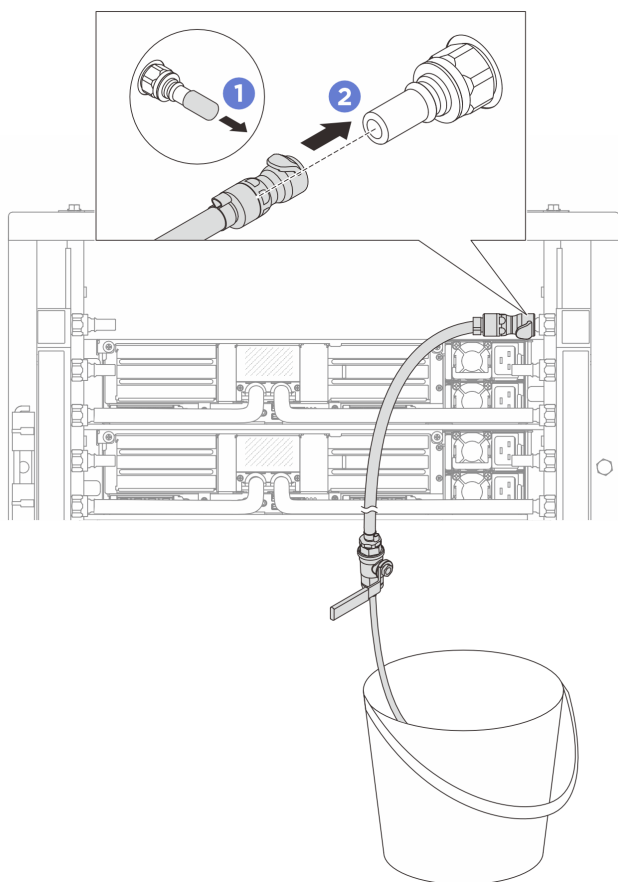
Рис. 147. Установка комплекта отводной трубки на стороне возврата
