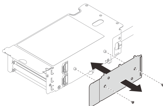
Рис. 177. Снятие кожуха кабелей
