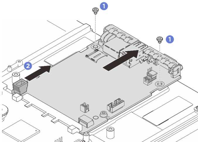
Рис. 225. Снятие системной платы ввода-вывода
