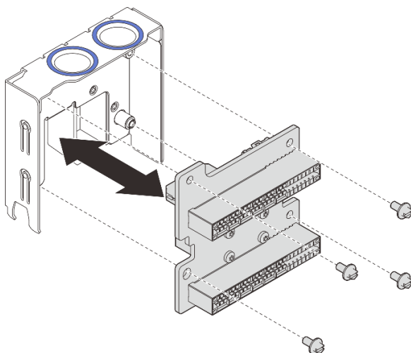
Рис. 186. Разборка платы распределения питания
