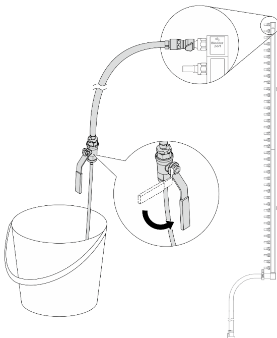
Рис. 139. Открытие клапана отводной трубы
