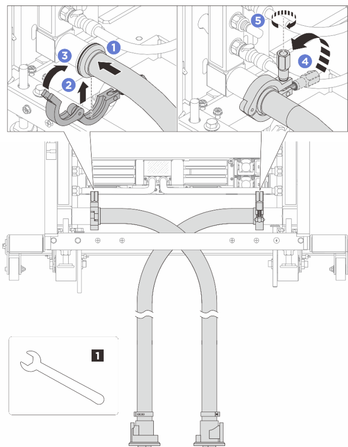
Рис. 143. Установка комплекта шланга
