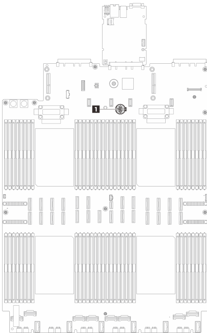
Рис. 22. Расположение гнезда батарейки CMOS
