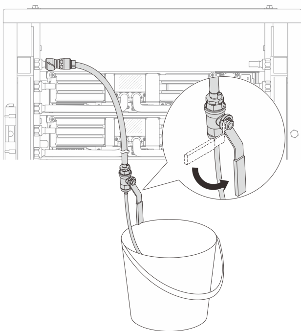
Рис. 129. Открытие клапана отводной трубки на стороне подачи
