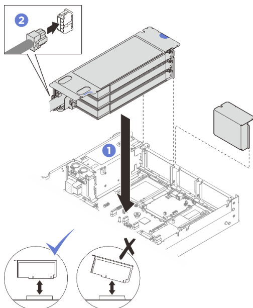
Рис. 171. Установка низкопрофильной платы-адаптера Riser PCIe (с разъемом питания)
