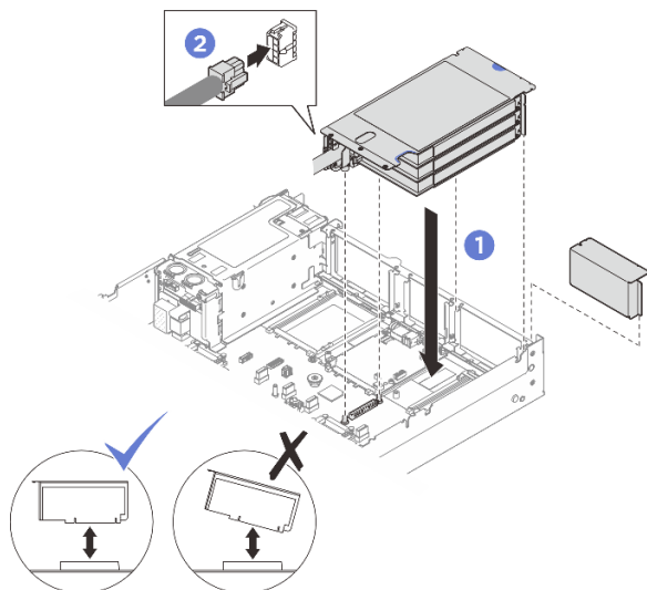
Рис. 172. Установка платы-адаптера Riser PCIe максимальной высоты, половинной длины
