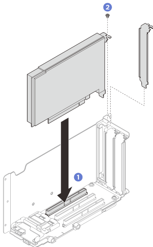
Рис. 167. Установка адаптера PCIe
