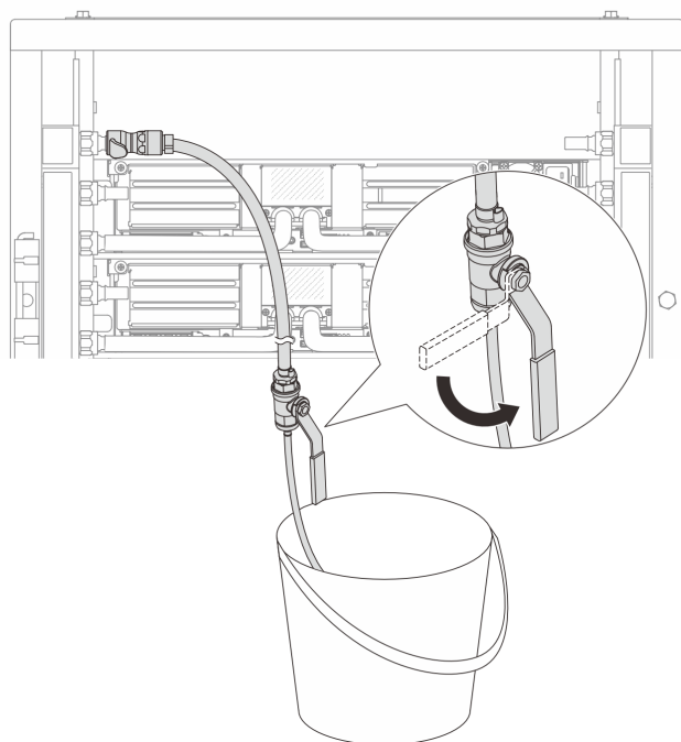
Рис. 150. Открытие клапана отводной трубки на стороне подачи
