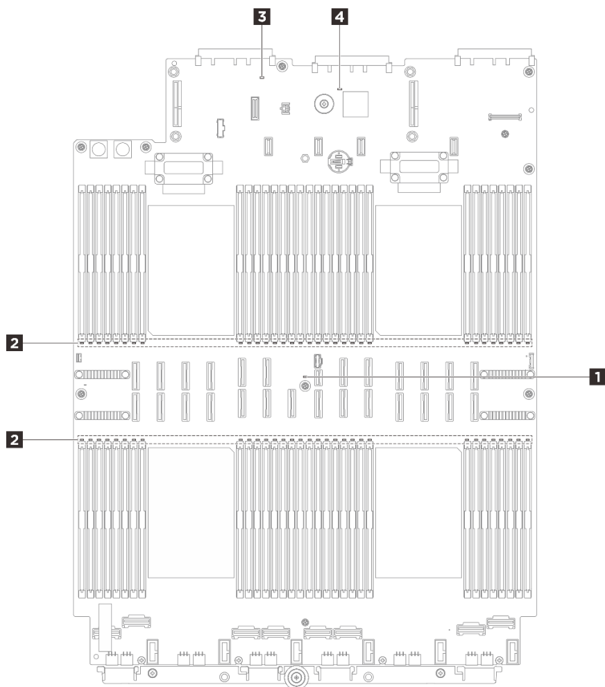
Рис. 254. Светодиодные индикаторы процессорной платы
