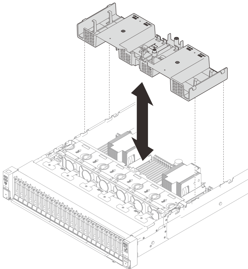
Рис. 11. Установка переднего дефлектора
