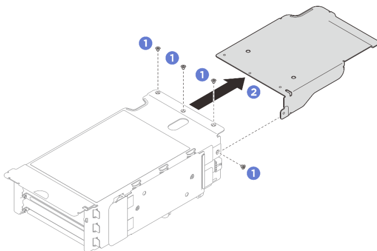
Рис. 183. Снятие расширителя платы-адаптера Riser PCIe
