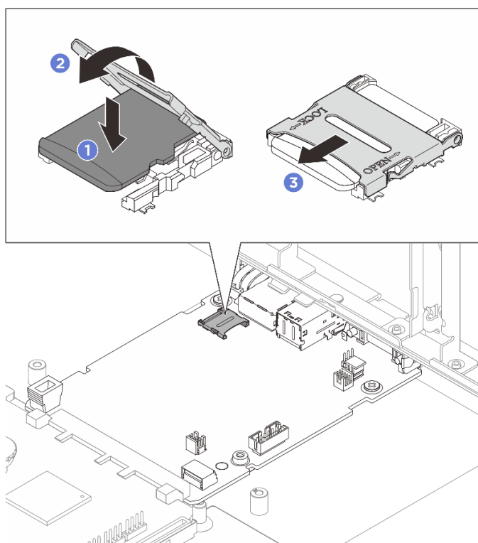
Рис. 157. Установка карты microSD
