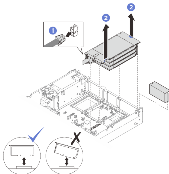
Рис. 164. Снятие платы-адаптера Riser PCIe максимальной высоты, половинной длины
