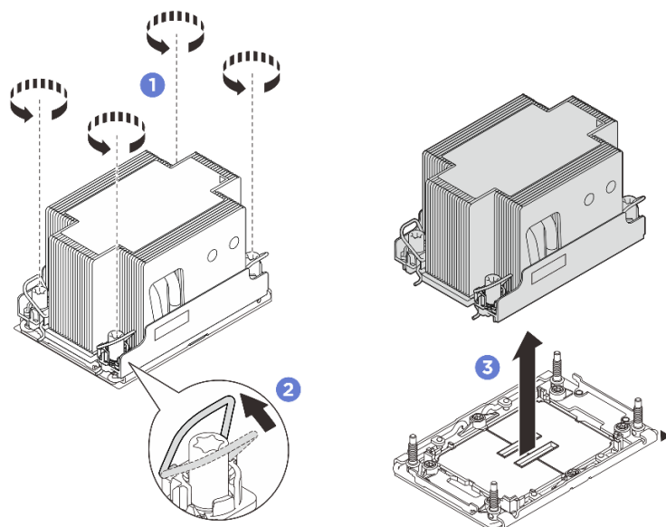
Рис. 191. Снятие стандартного модуля PHM 2U
