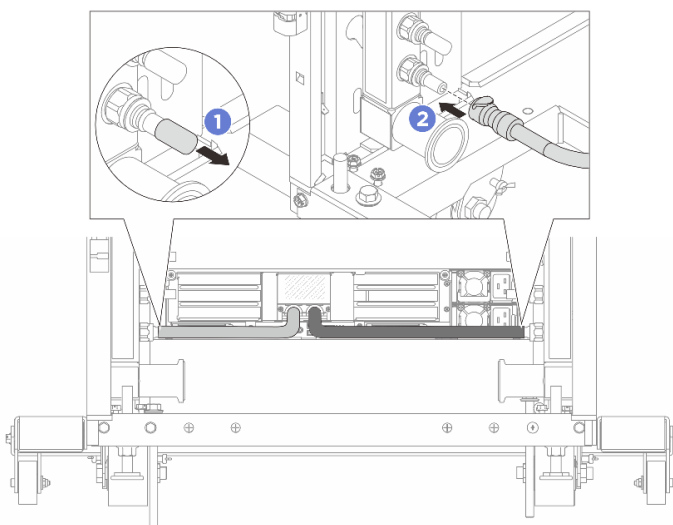
Рис. 126. Установка быстроразъемного соединителя
