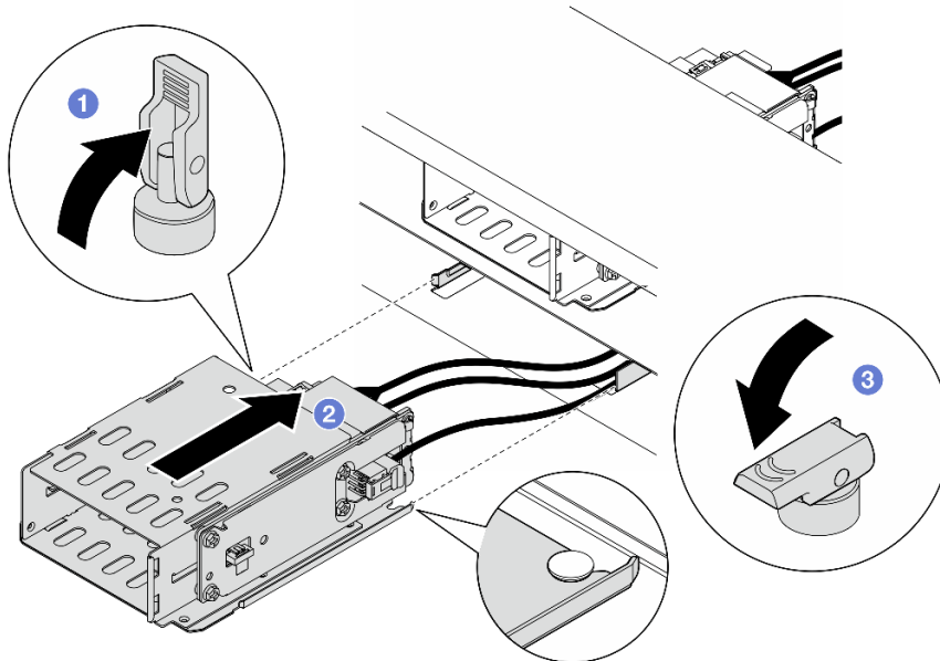
Рис. 36. Установка отсека E3.S 2T
