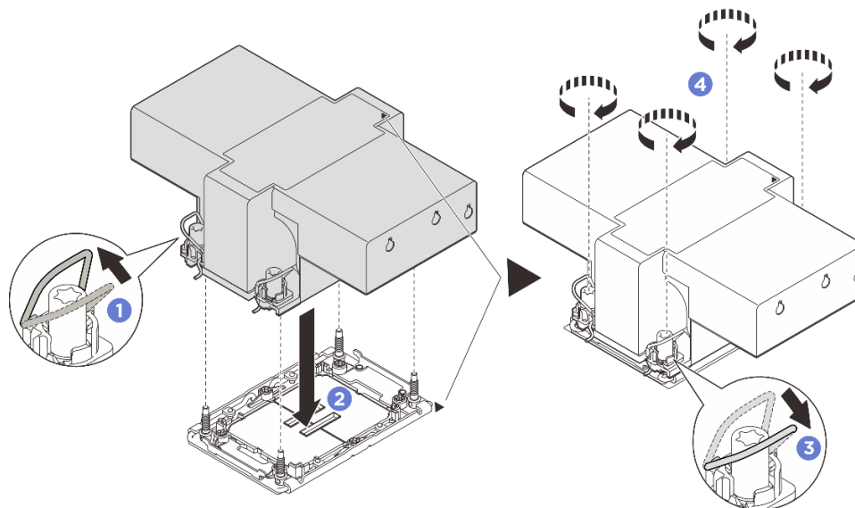
Рис. 200. Установка модуля PNM повышенной мощности 2U
