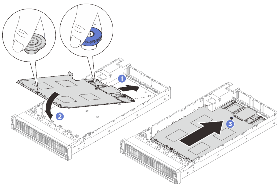
Рис. 227. Установка блока материнской платы
