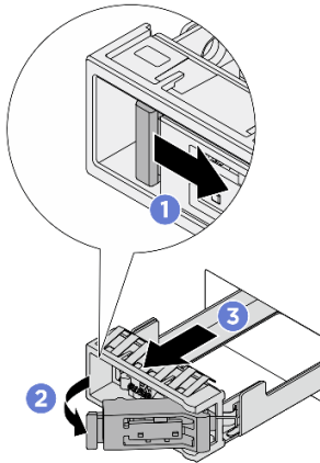
Рис. 73. Снятие лотка для дисков M.2
