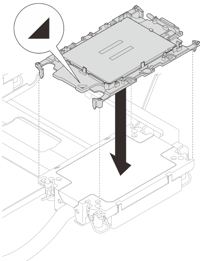
Рис. 87. Установка процессора на плату охлаждения
