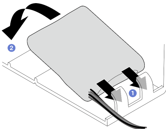
Рис. 56. Установка модуля питания флэш-памяти
