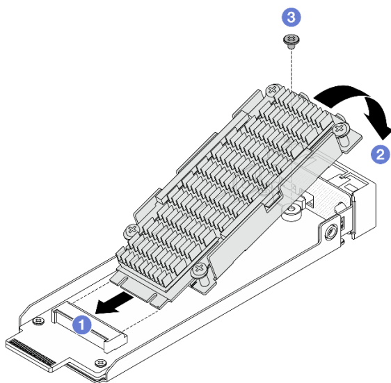
Рис. 72. Установка диска M.2 с радиатором
