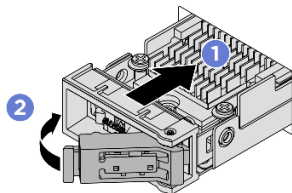
Рис. 74. Установка блока дисков M.2
