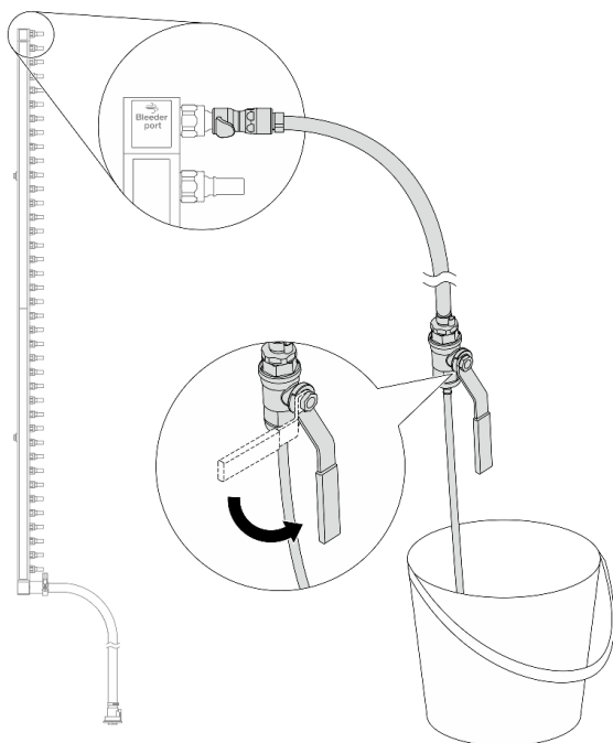
Рис. 137. Открытие клапана отводной трубки
