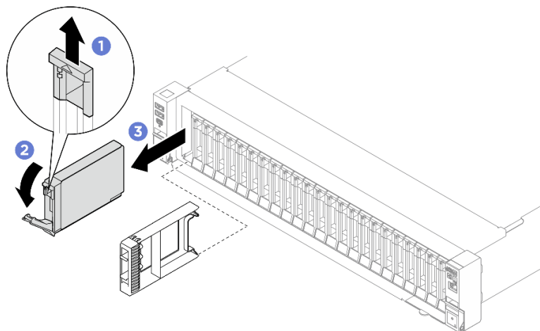
Рис. 4. Снятие 2,5-дюймового оперативно заменяемого диска
