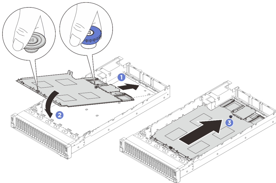
Рис. 231. Установка блока материнской платы
