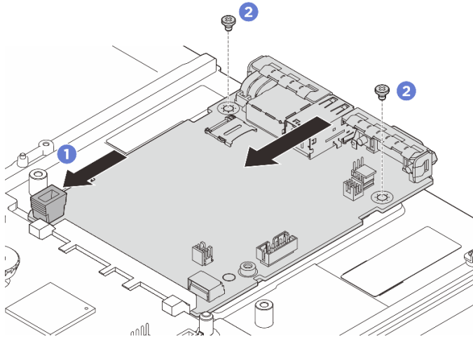
Рис. 230. Установка системной платы ввода-вывода
