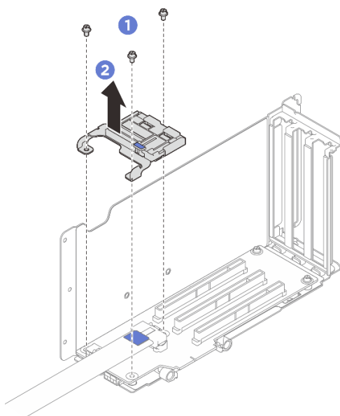
Рис. 181. Снятие фиксатора PCIe
