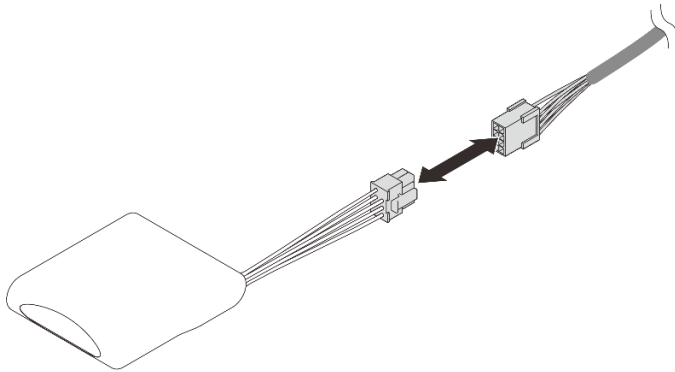
Рис. 53. Отключение кабеля модуля питания флэш-памяти
