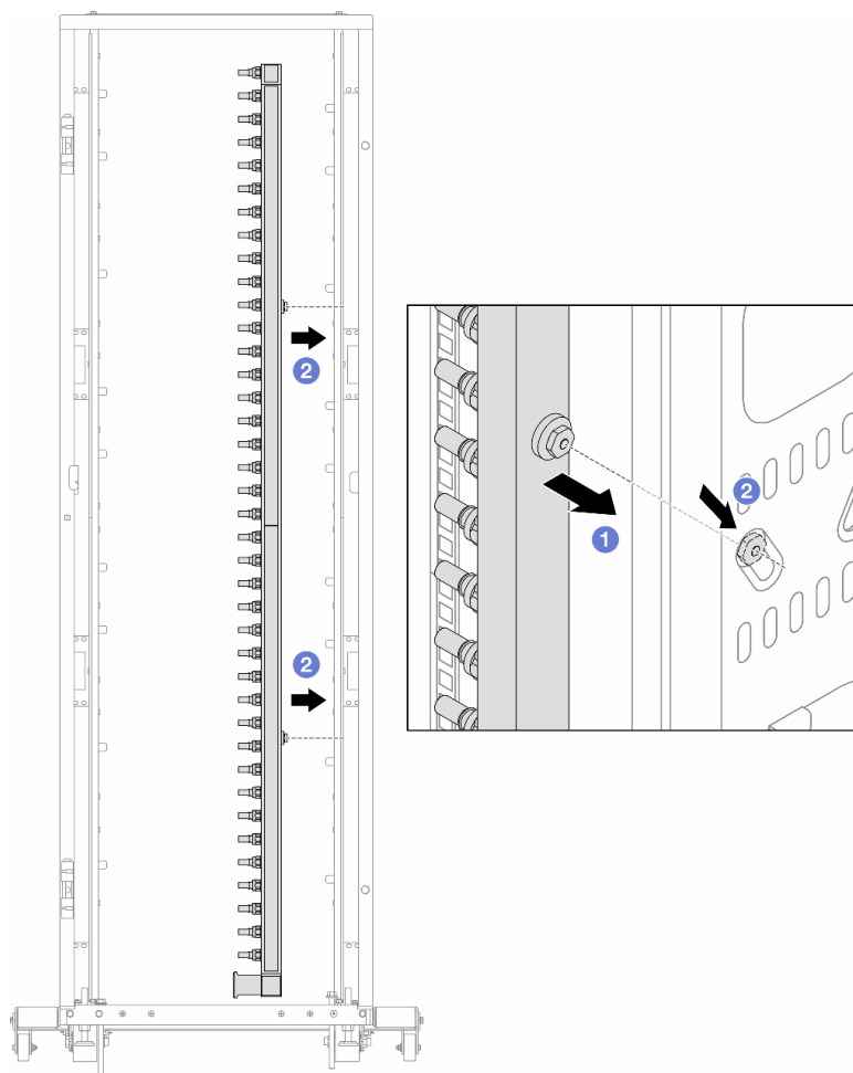
Рис. 141. Установка коллектора
