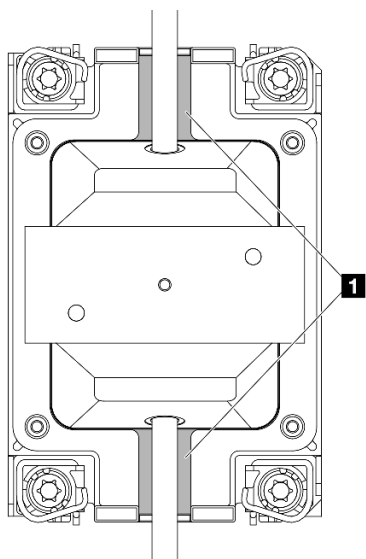
Рис. 257. Области, подверженные возникновению утечек
