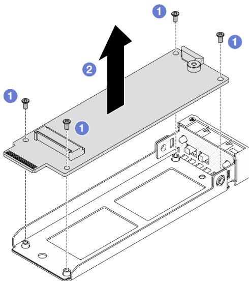
Рис. 66. Снятие интерпозера M.2
