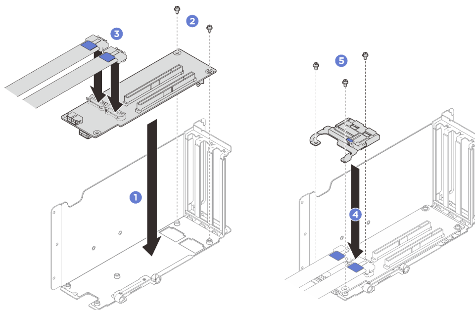
Рис. 178. Установка платы-адаптера Riser PCIe
