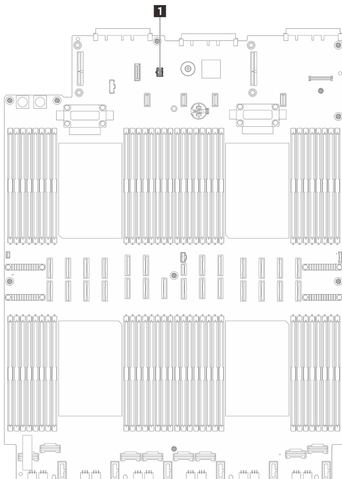
Рис. 95. Подключение модуля датчика обнаружения утечки
