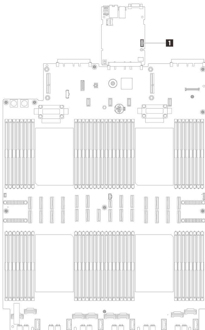
Рис. 220. Расположение разъема последовательного порта
