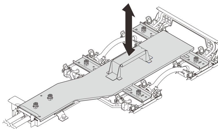
Рис. 92. Снятие держателя платы охлаждения
