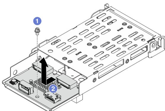
Рис. 208. Снятие адаптера загрузки M.2
