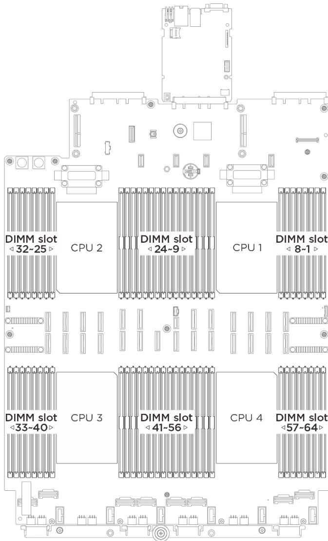
Рис. 152. Расположение модулей памяти и процессоров
