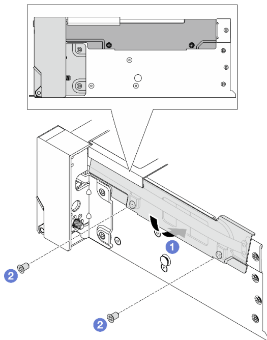
Рис. 206. Установка фиксатора кабелей
