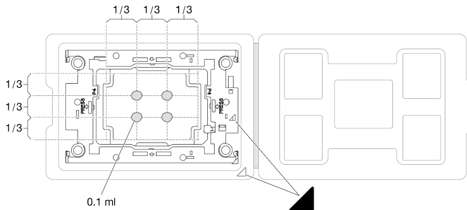
Рис. 86. Нанесение термопасты на процессор в транспортировочном лотке
