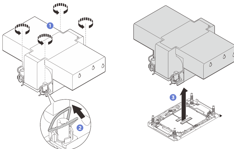
Рис. 192. Снятие модуля РНМ повышенной мощности 2U
