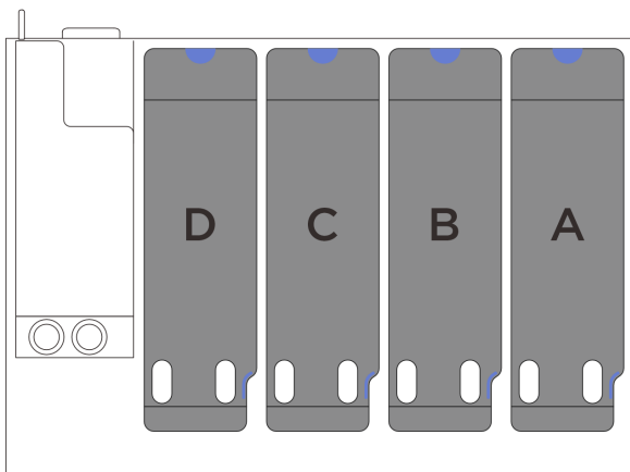
Рис. 162. модели серверов с четырьмя платами-адаптерами Riser PCIe
