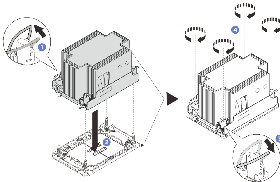
Рис. 199. Установка стандартного модуля PNM 2U
