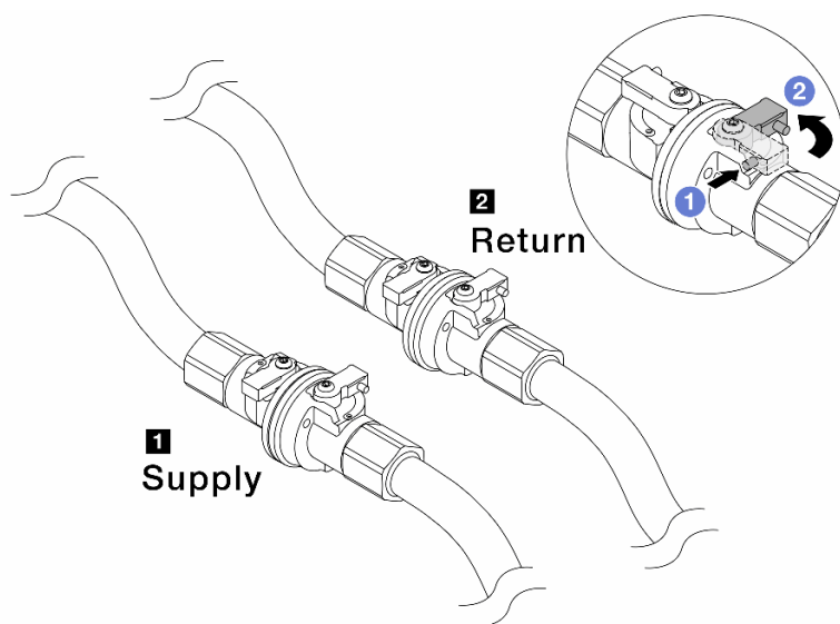
Рис. 133. Закрытие шаровых клапанов
