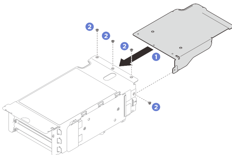
Рис. 184. Установка расширителя платы-адаптера Riser PCIe
