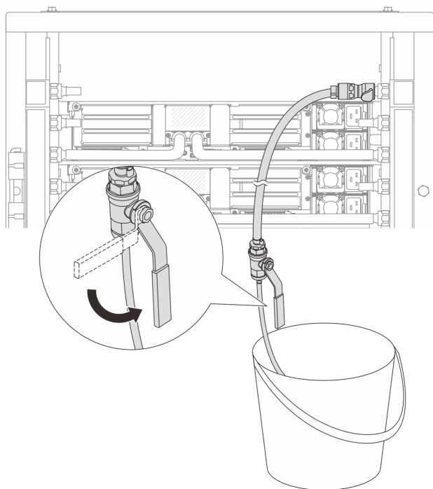
Рис. 131. Открытие клапана отводной трубки на стороне возврата
