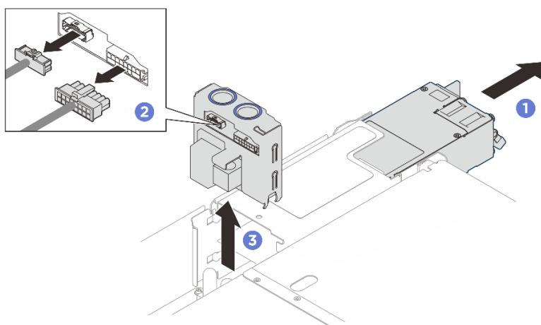
Рис. 185. Снятие платы распределения питания
