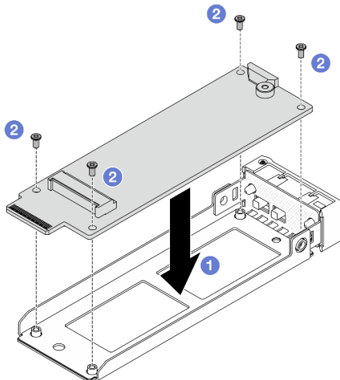
Рис. 71. Установка интерпозера M.2
