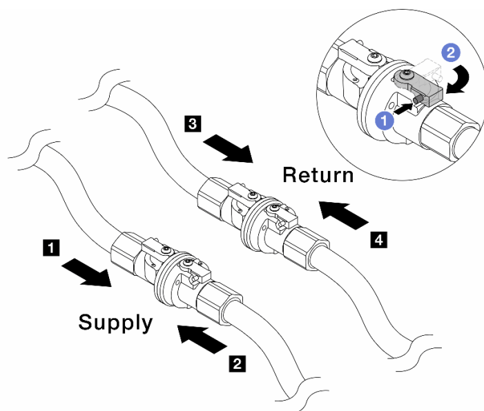
Рис. 151. Открытие шаровых клапанов
