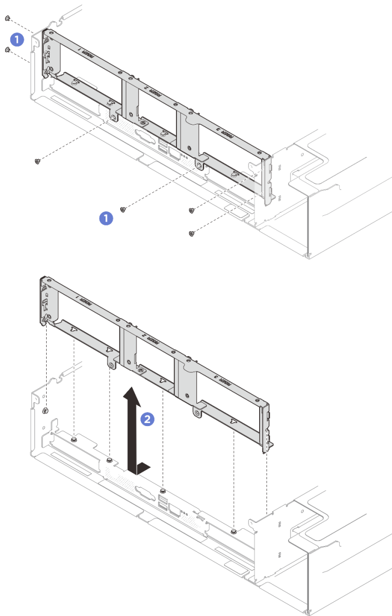
Рис. 211. Снятие задней стенки
