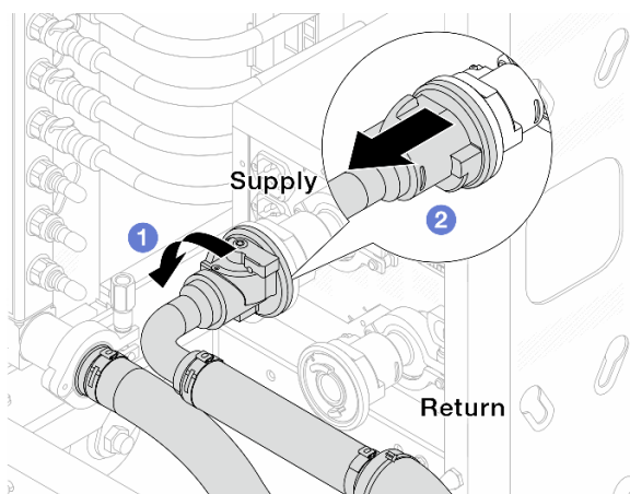
Рис. 112. Снятие комплекта соединений
