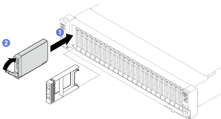
Рис. 7. Установка 2,5-дюймового оперативно заменяемого диска
