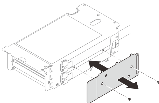
Рис. 180. Установка кожуха кабелей
