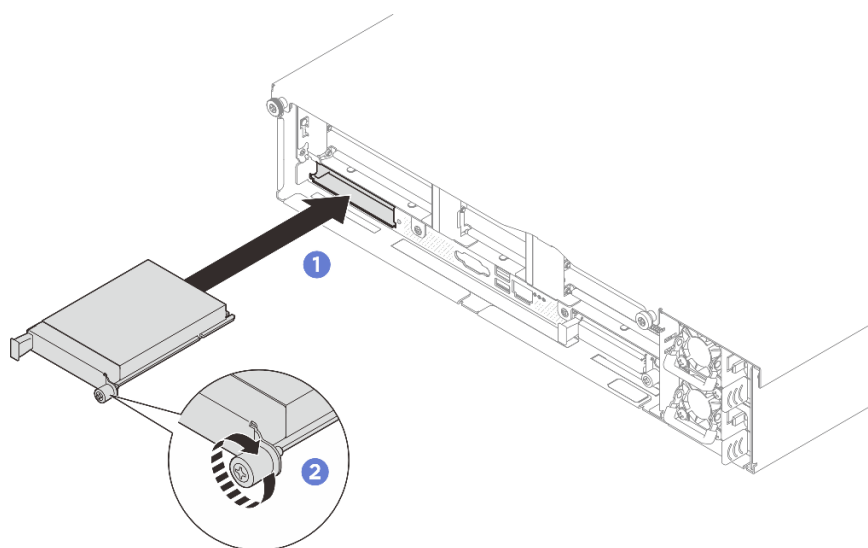
Рис. 159. Установка модуля OCP
