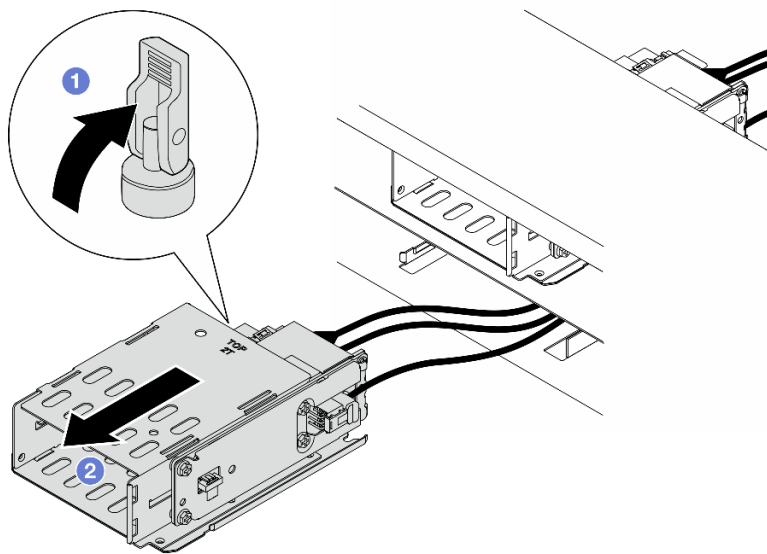
Рис. 33. Снятие отсека E3.S 2T
