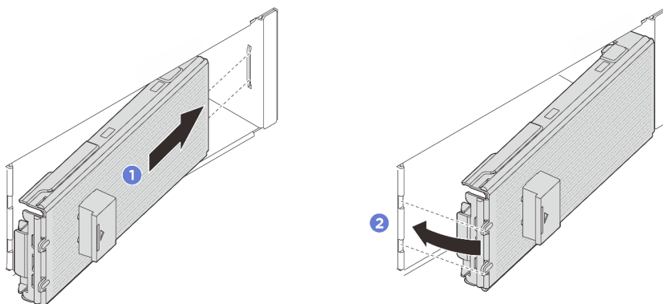
Рис. 44. Установка панели E3.S
