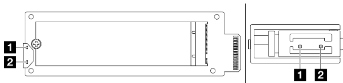
Рис. 251. Светодиодные индикаторы заднего интерпозера M.2
