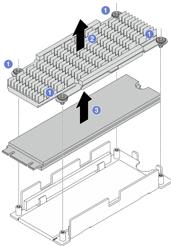
Рис. 67. Отделение диска M.2 и радиатора
