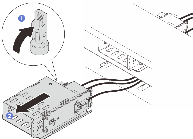
Рис. 45. Снятие отсека E3.S 1T
