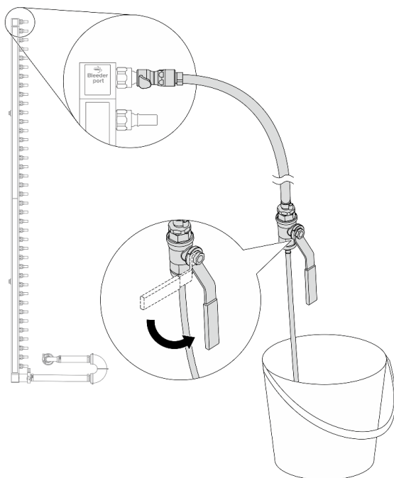
Рис. 115. Открытие клапана отводной трубки
