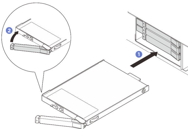
Рис. 41. Установка оперативно заменяемого диска E3.S
