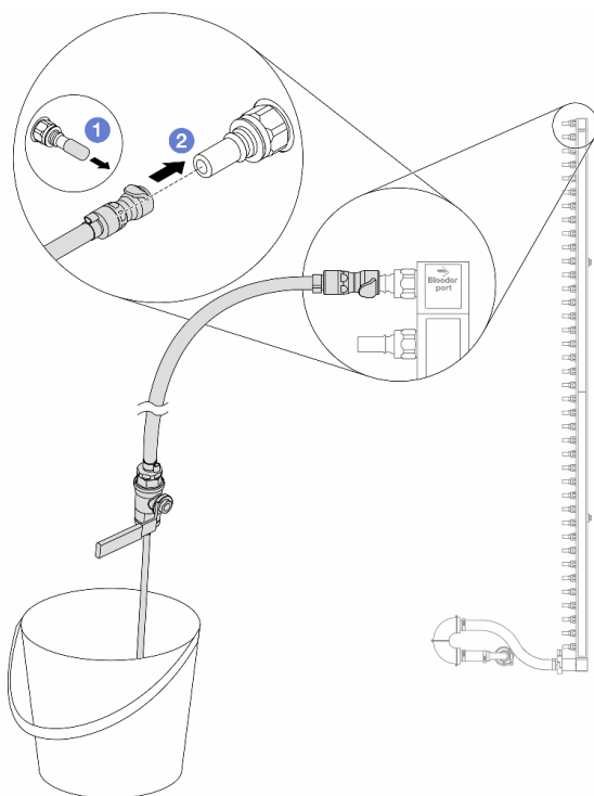
Рис. 116. Установка комплекта отводной трубки на стороне возврата
