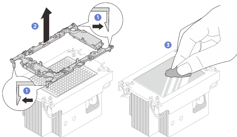
Рис. 194. Снятие держателя процессора с радиатора
