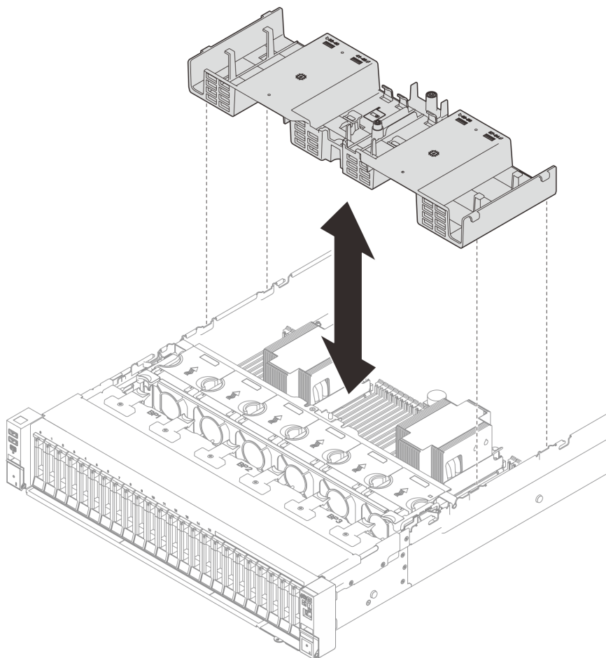
Рис. 10. Снятие переднего дефлектора
