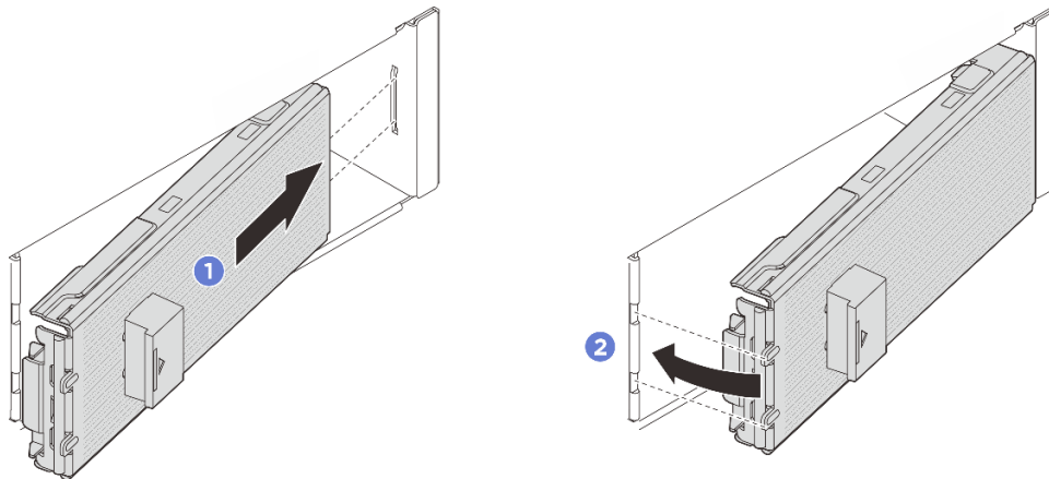
Рис. 32. Установка панели E3.S
