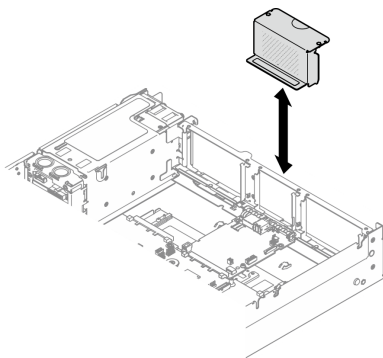
Рис. 78. Снятие заглушки платы-адаптера Riser
