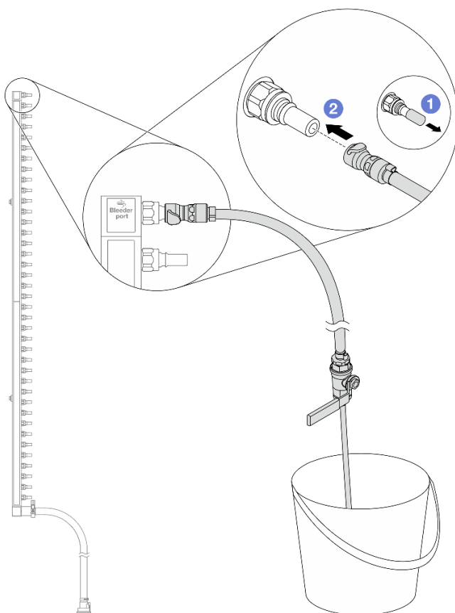
Рис. 136. Установка комплекта отводной трубки на стороне подачи
