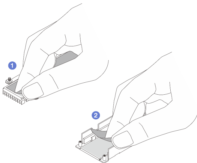
Рис. 69. Снятие пленок
