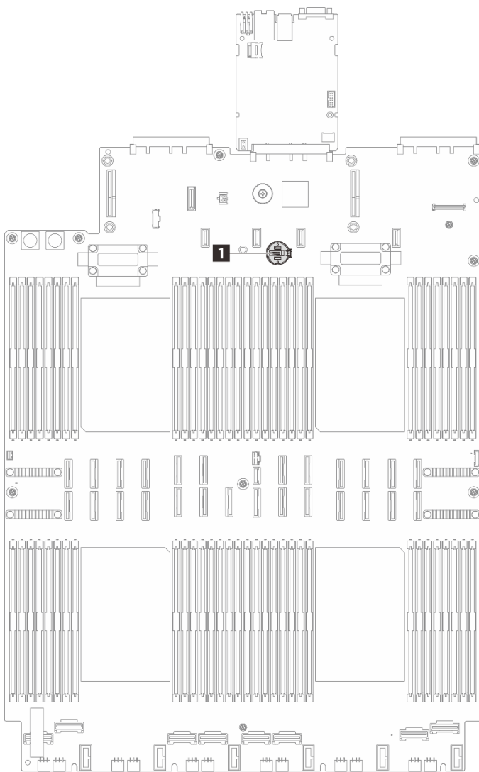
Рис. 20. Расположение батарейки CMOS
