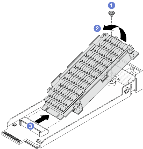
Рис. 65. Снятие диска M.2 с радиатором
