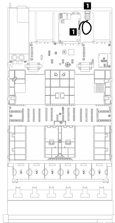
Рис. 222. Прокладка кабеля для модуля последовательного порта для модели сервера с четырьмя платами-адаптерами Riser PCIe
