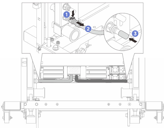
Рис. 111. Отсоединение быстроразъемного соединителя
