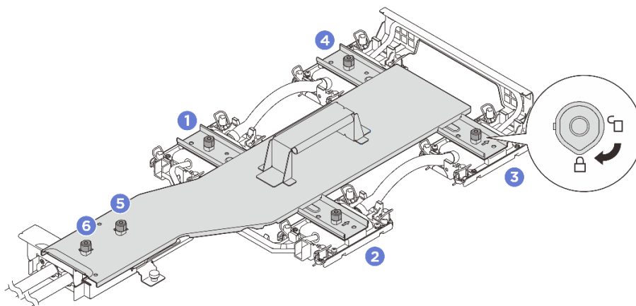
Рис. 81. Крепление держателя платы охлаждения
