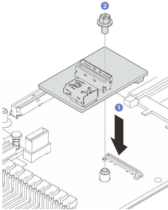
Рис. 239. Установка платы ввода-вывода USB
