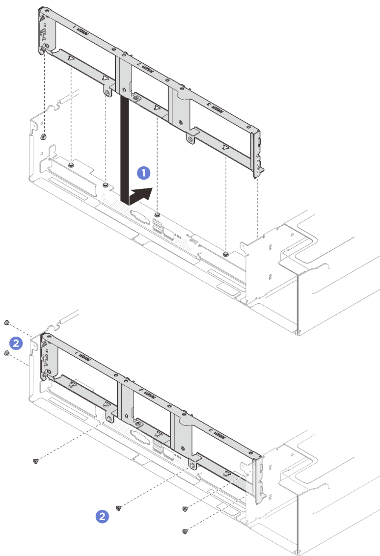
Рис. 212. Установка задней стенки
