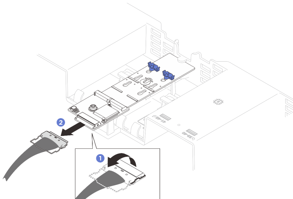
Рис. 15. Отключение кабеля адаптера загрузки M.2
