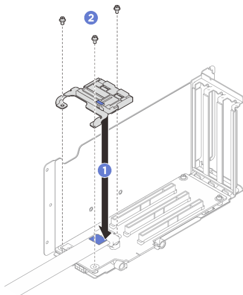
Рис. 182. Установка фиксатора PCIe
