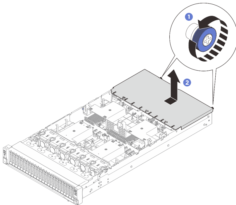
Рис. 234. Снятие заднего верхнего кожуха
