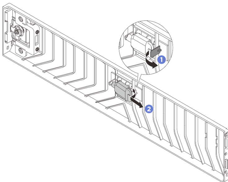
Рис. 215. Снятие ключа
