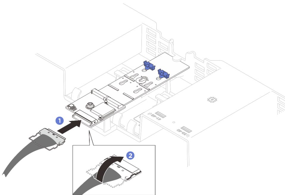
Рис. 18. Подключение кабелей адаптера загрузки M.2
