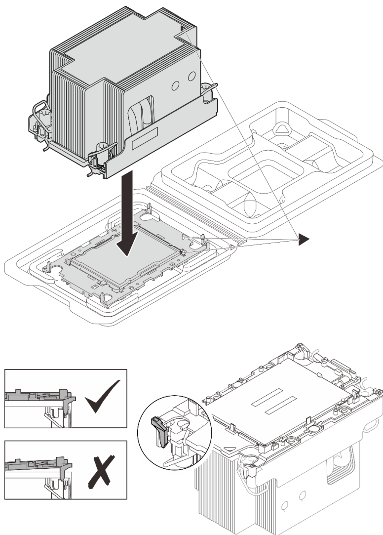
Рис. 198. Сборка модуля процессора с радиатором (PHM), когда процессор находится в транспортировочной лотке
