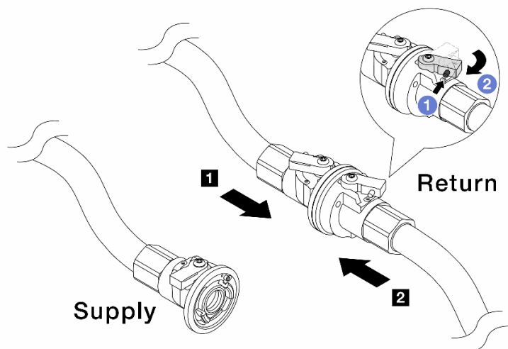
Рис. 145. Подключение разъема на стороне подачи объекта к разъему на стороне возврата коллектора
