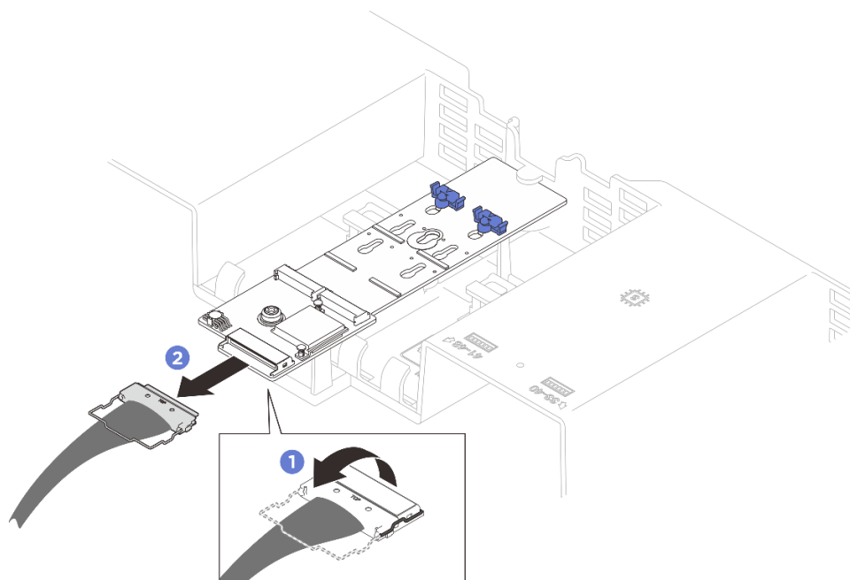
Рис. 97. Отключение кабеля адаптера загрузки M.2
