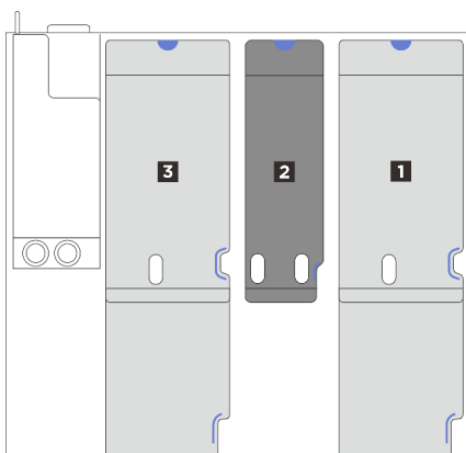
Рис. 169. Модели серверов с тремя платами-адаптерами Riser PCIe и расширителями платы-адаптера Riser
