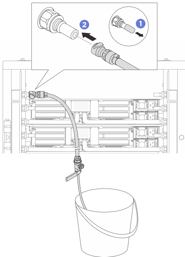
Рис. 127. Установка комплекта отводной трубки на стороне подачи
