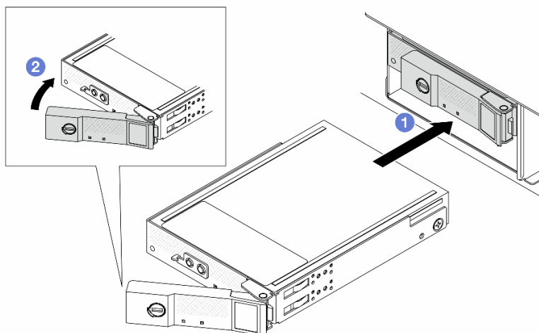
Рис. 29. Установка СММ E3.S
