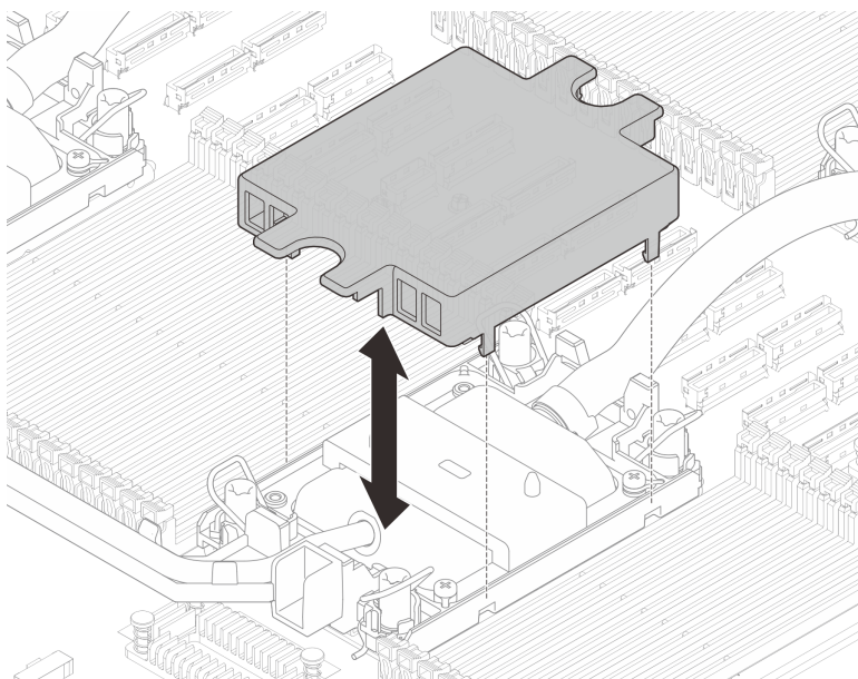
Рис. 79. Снятие кожухов платы охлаждения
