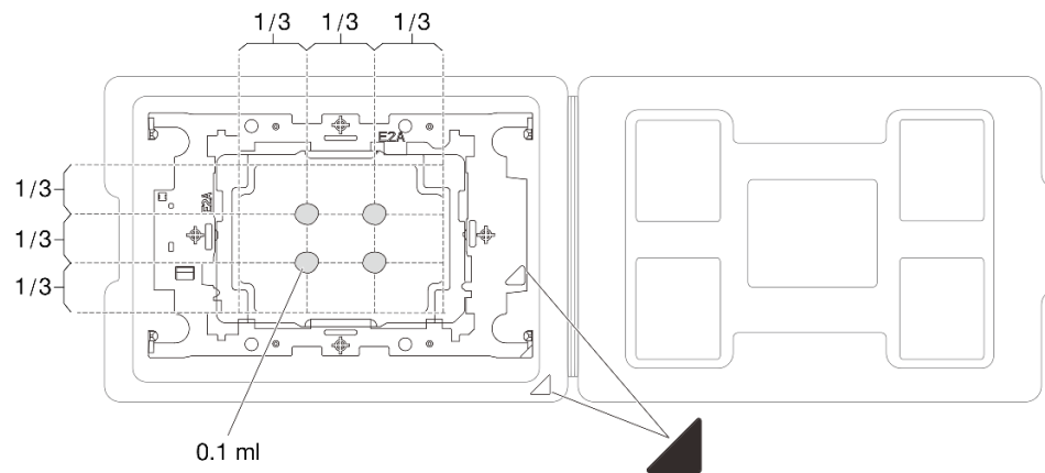
Рис. 197. Нанесение термопасты на процессор в транспортировочном лотке
