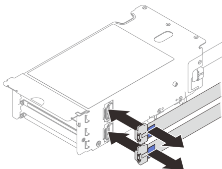
Рис. 175. Отключение кабелей
