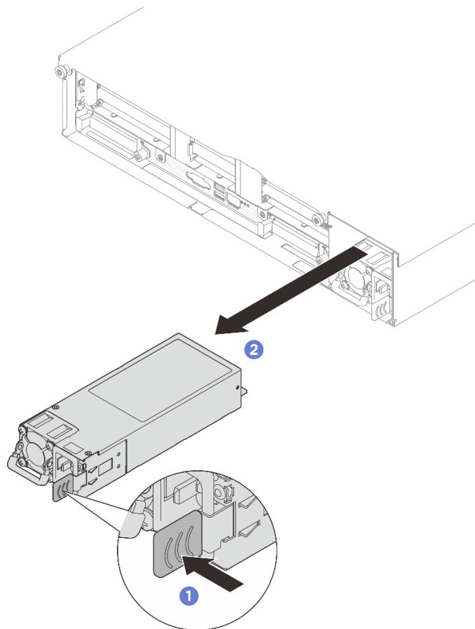
Рис. 188. Снятие блока питания
