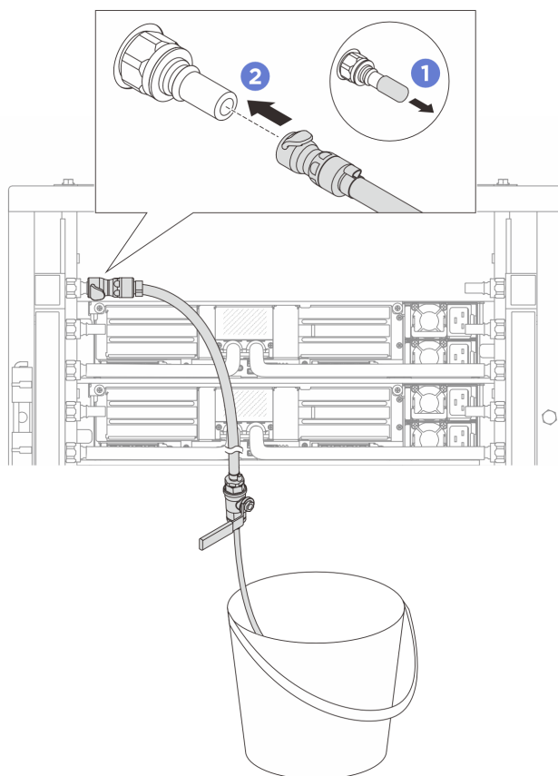
Рис. 144. Установка комплекта отводной трубы на стороне подачи
