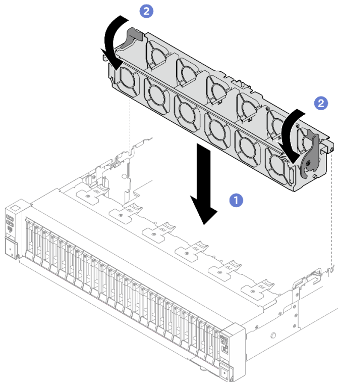
Рис. 51. Установка отсека вентиляторов
