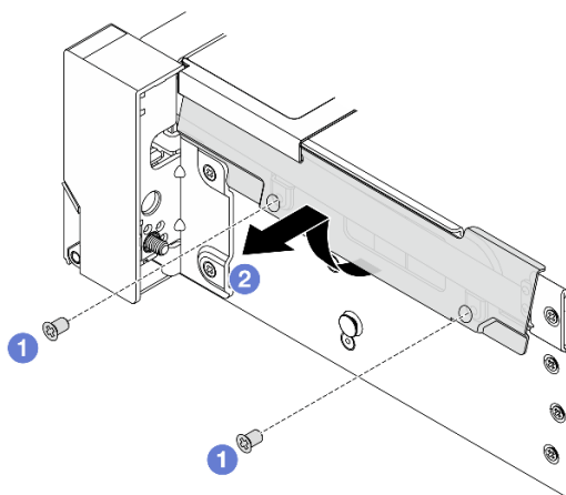
Рис. 201. Снятие фиксатора кабелей
