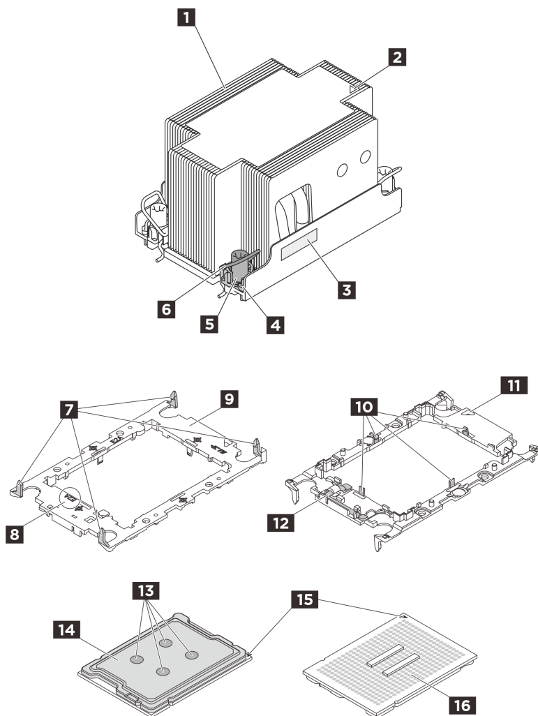
Рис. 195. Компоненты PBM
