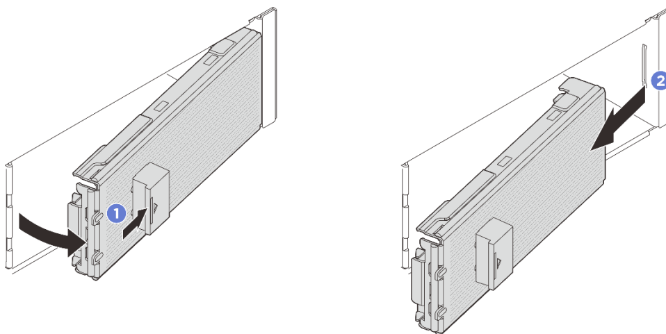
Рис. 27. Снятие панели E3.S
