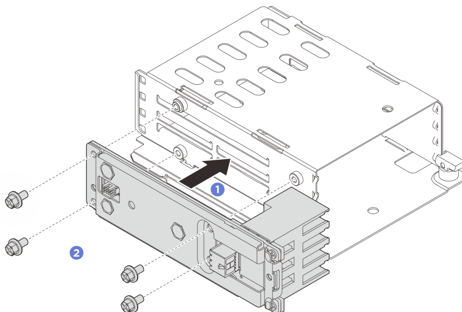
Рис. 47. Установка блока объединительной панели
