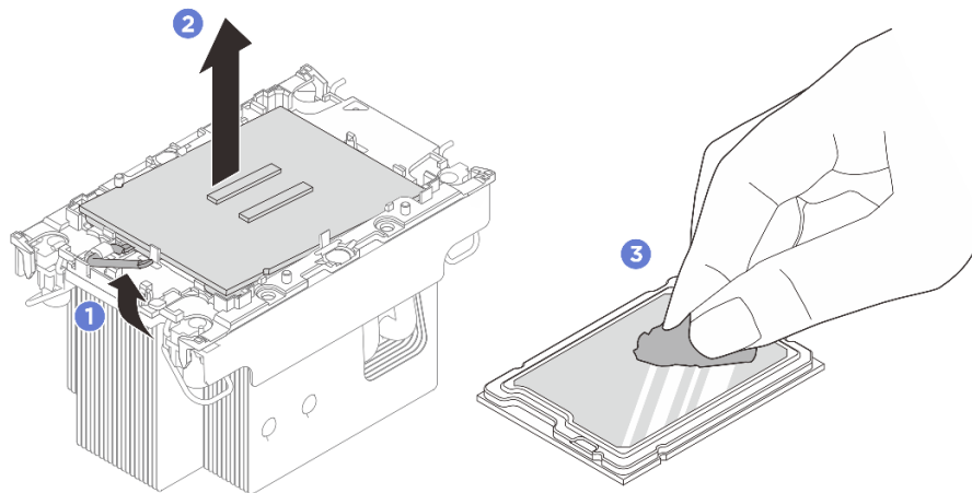
Рис. 193. Отделение процессора от радиатора и держателя
