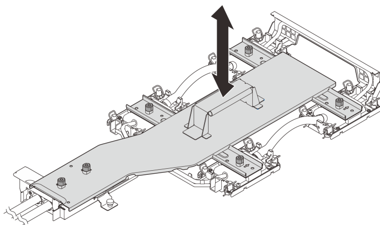
Рис. 80. Установка держателя платы охлаждения
