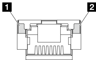
Рис. 256. Светодиодные индикаторы на Порт управления системой ХСС (RJ-45 10/100/1000 Мбит/с)
