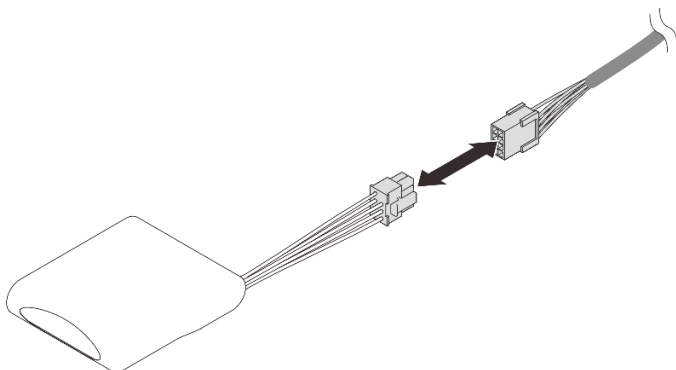
Рис. 13. Подключение кабеля модуля питания флэш-памяти
