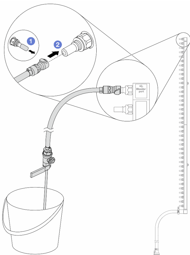
Рис. 138. Установка комплекта отводной трубки на стороне возврата
