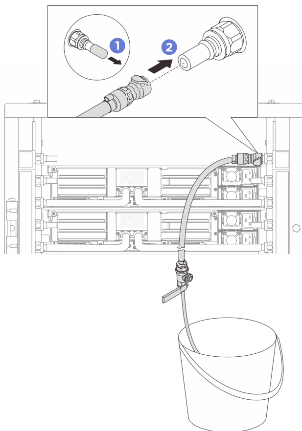
Рис. 130. Установка комплекта отводной трубки на стороне возврата
