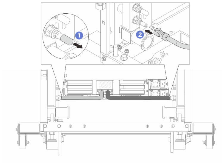
Рис. 142. Установка быстроразъемного соединителя
