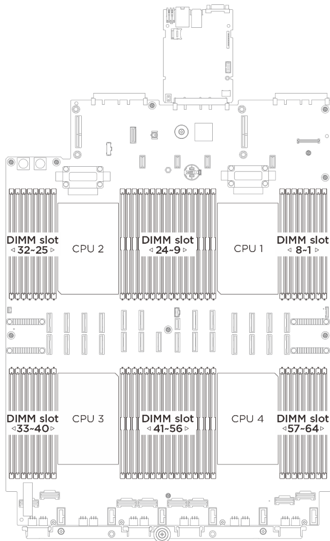
Рис. 154. Расположение модулей памяти и процессоров
