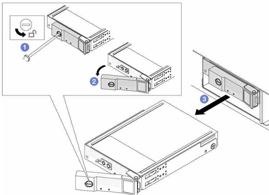
Рис. 25. Снятие СММ
