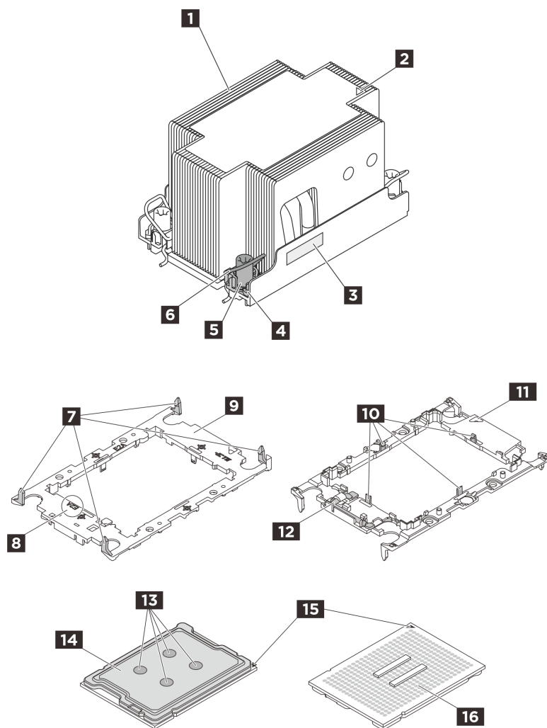
Рис. 190. Компоненты PNM
