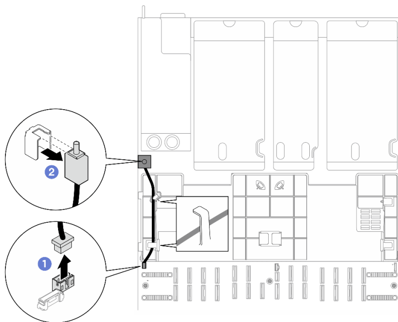
Рис. 75. Снятие датчика вмешательства
