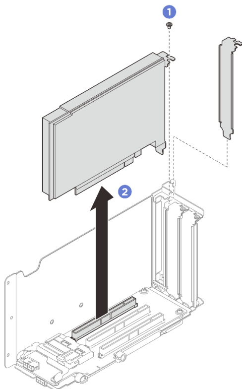
Рис. 166. Снятие адаптера PCIe
