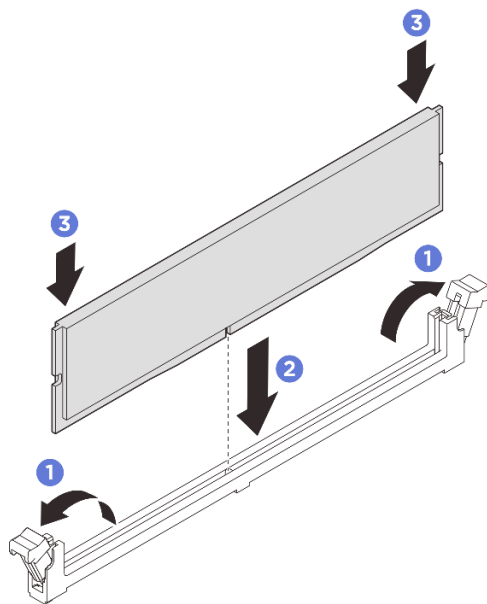
Рис. 155. Установка модуля памяти
