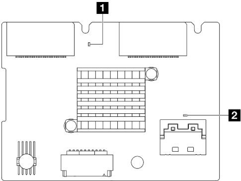
Рис. 252. Светодиодные индикаторы заднего адаптера загрузки M.2
