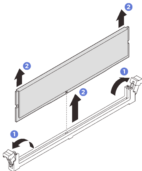
Рис. 153. Снятие модуля памяти
