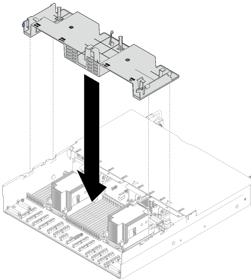
Рис. 17. Установка заднего дефлектора
