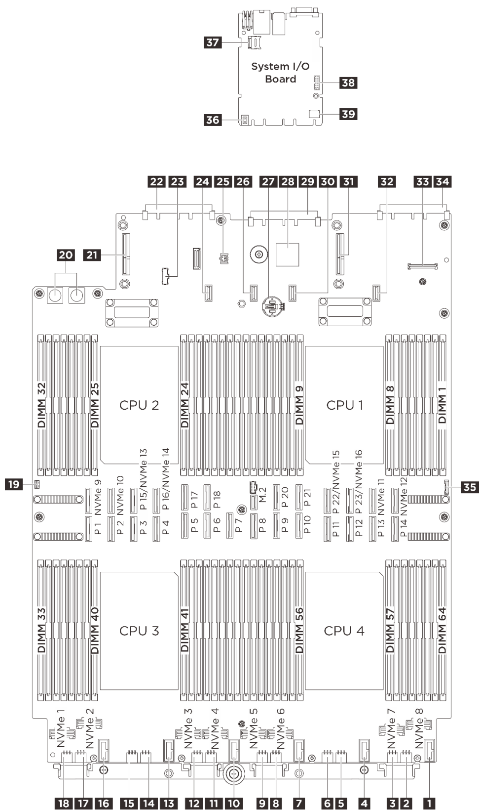
Рис. 242. Разъемы блока материнской платы
