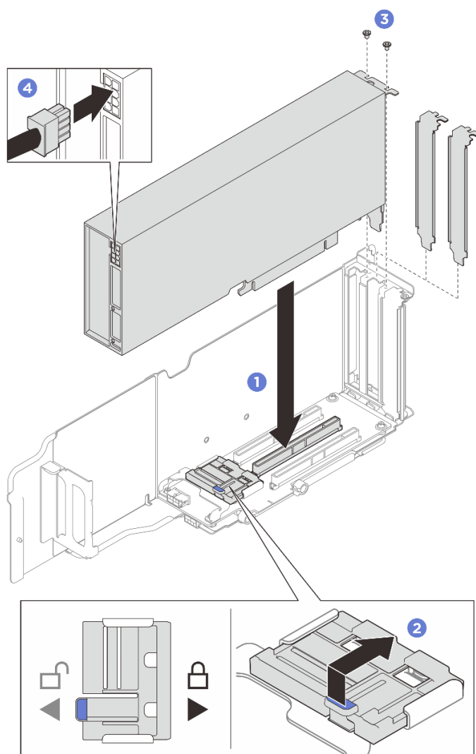
Рис. 61. Установка адаптера графического процессора двойной ширины
