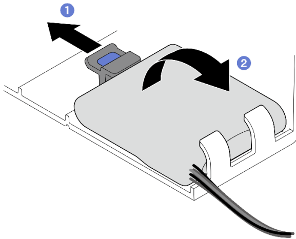
Рис. 54. Снятие модуля питания флэш-памяти
