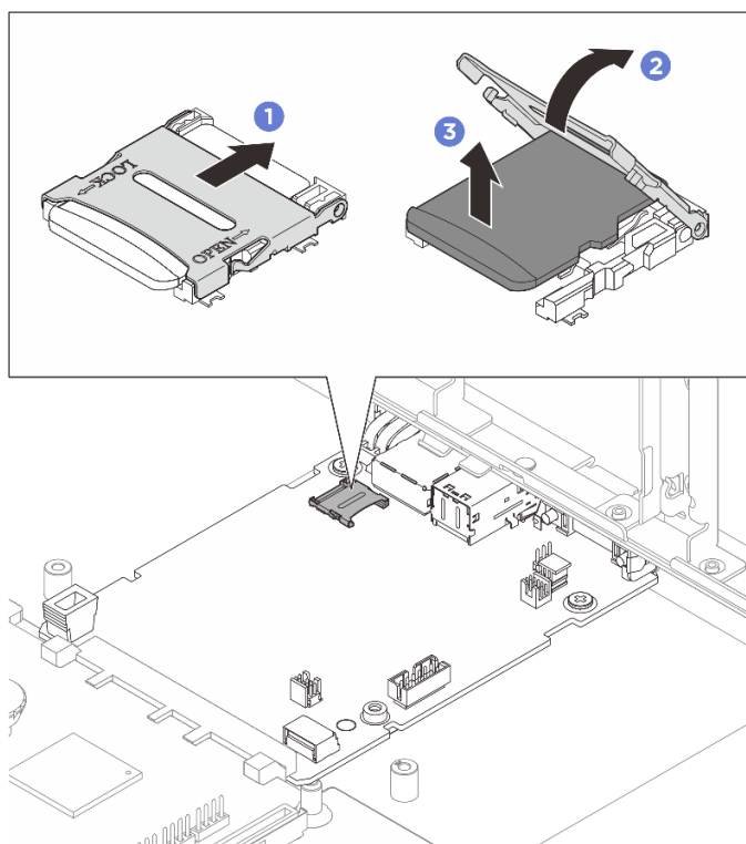
Рис. 156. Извлечение карты microSD
