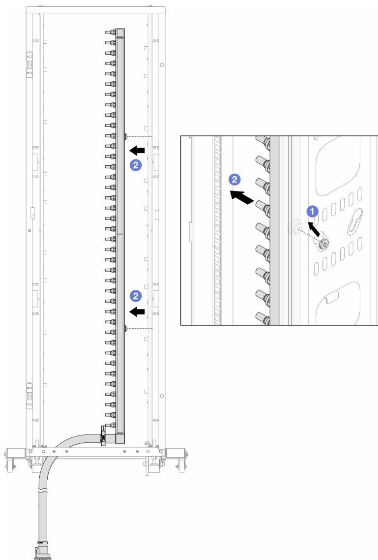
Рис. 135. Снятие коллектора
