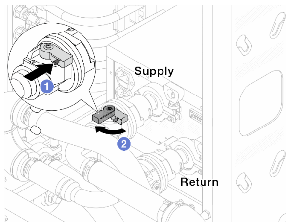
Рис. 128. Открытие шаровых клапанов
