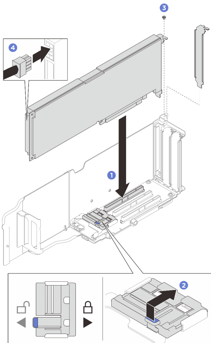
Рис. 60. Установка адаптера графического процессора одинарной ширины
