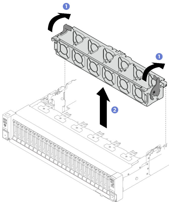
Рис. 50. Снятие отсека вентиляторов
