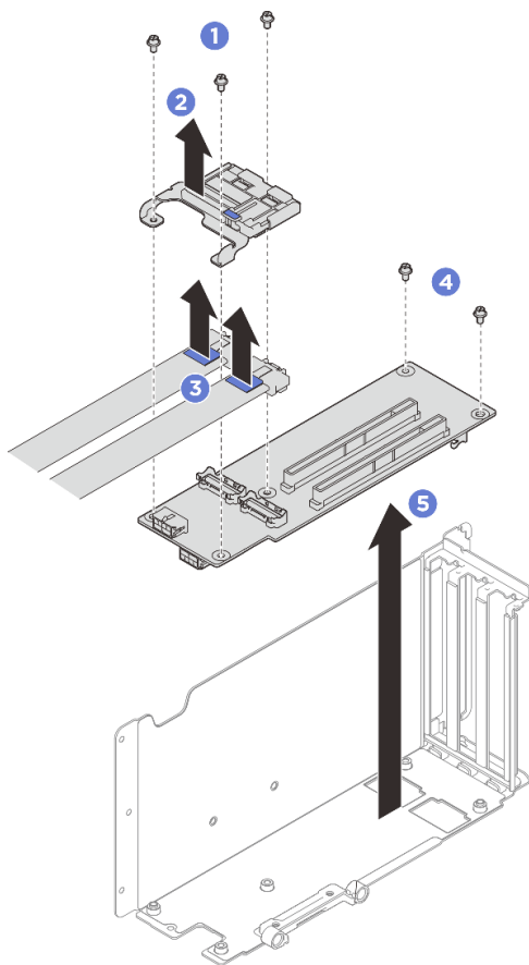
Рис. 176. Снятие платы-адаптера Riser PCIe
