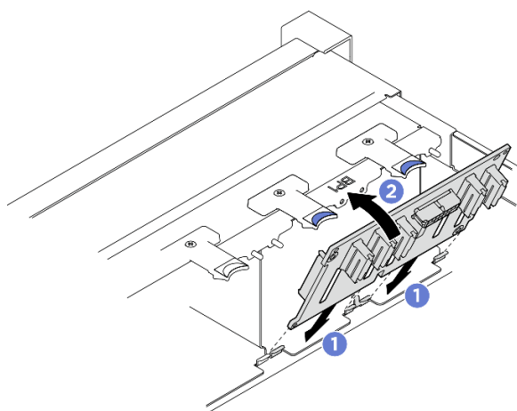
Рис. 6. Установка объединительной панели 2,5-дюймовых дисков
