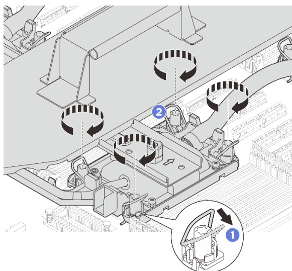
Рис. 90. Затяжка гаек Torx T30
