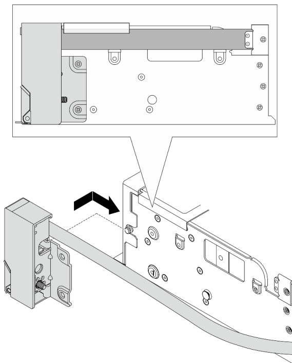
Рис. 204. Установка защелки стойки
