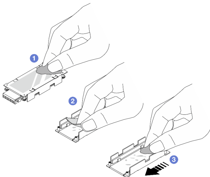
Рис. 68. Очистка радиатора и нижней пластины
