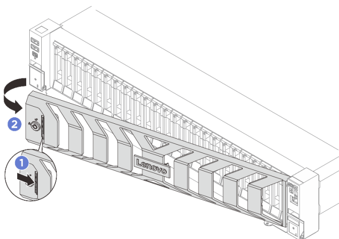
Рис. 214. Снятие защитной панели
