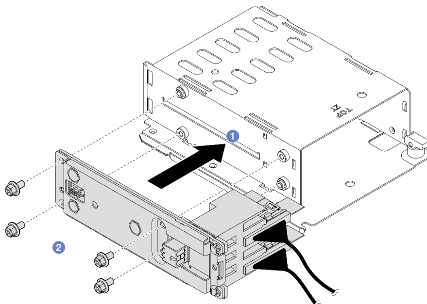
Рис. 35. Установка объединительной панели
