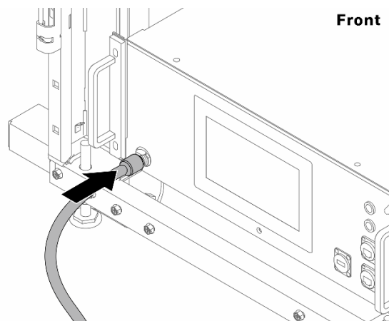
Рис. 124. Передняя сторона блока CDU
