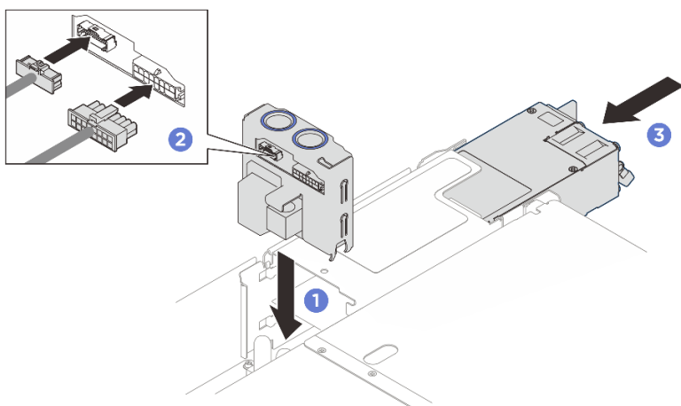
Рис. 187. Установка платы распределения питания
