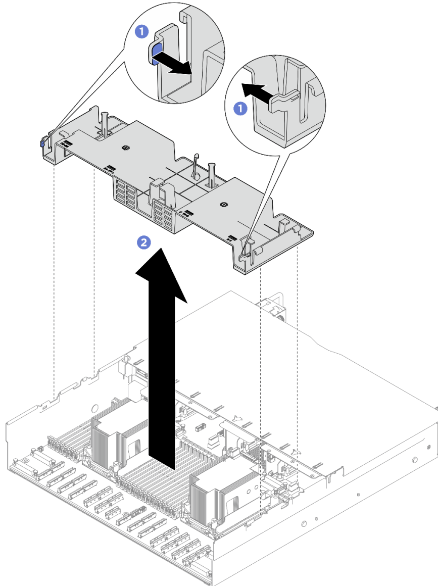
Рис. 16. Снятие заднего дефлектора
