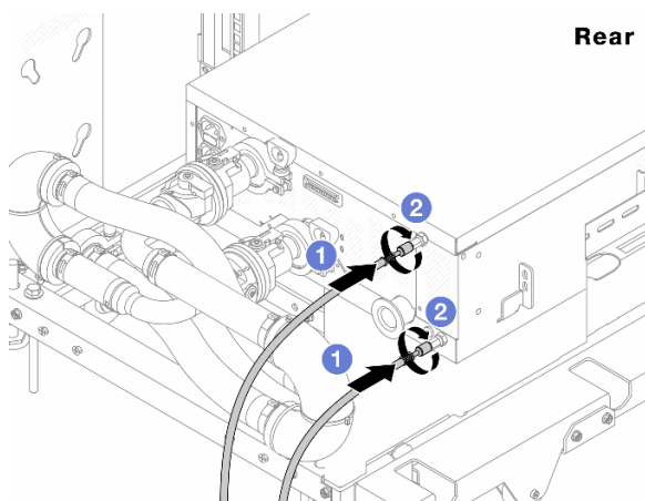
Рис. 125. Задняя сторона блока CDU
