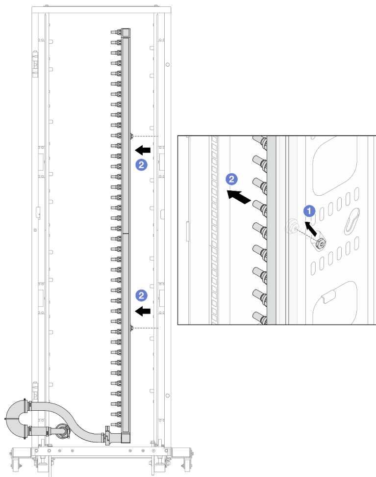
Рис. 113. Снятие коллектора
