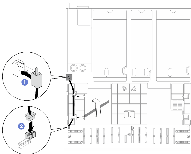
Рис. 76. Установка датчика вмешательства
