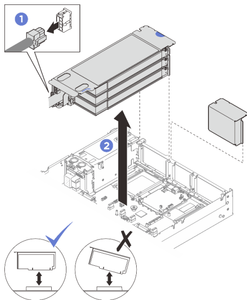
Рис. 163. Снятие низкопрофильной платы-адаптера Riser PCIe (с разъемом питания)
