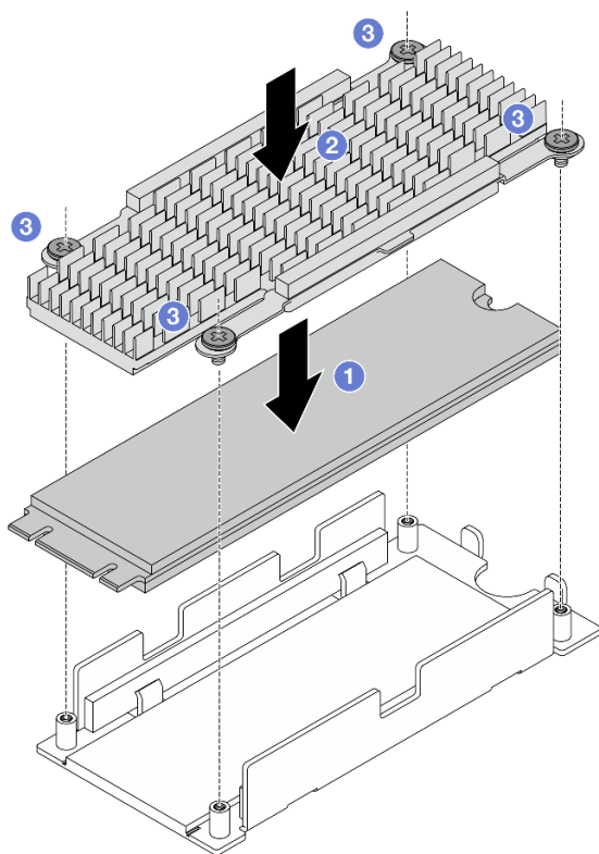
Рис. 70. Сборка радиатора и диска M.2
