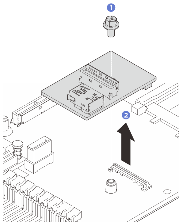
Рис. 238. Снятие платы ввода-вывода USB
