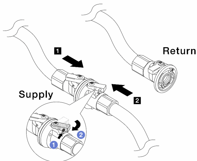
Рис. 148. Подключение разъема на стороне подачи объекта к разъему на стороне подачи коллектора
