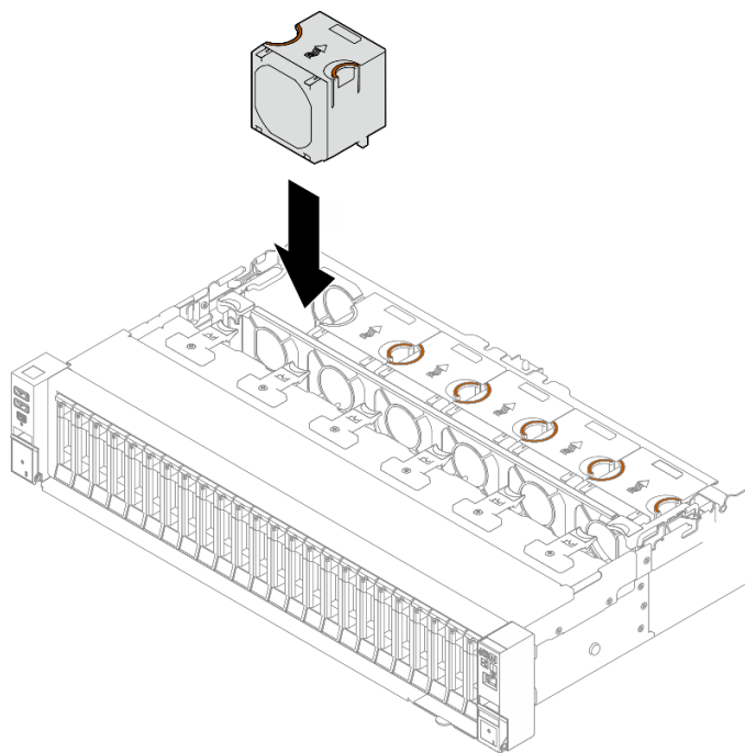
Рис. 52. Установка вентилятора
