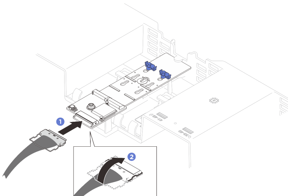
Рис. 12. Подключение кабелей адаптера загрузки M.2
