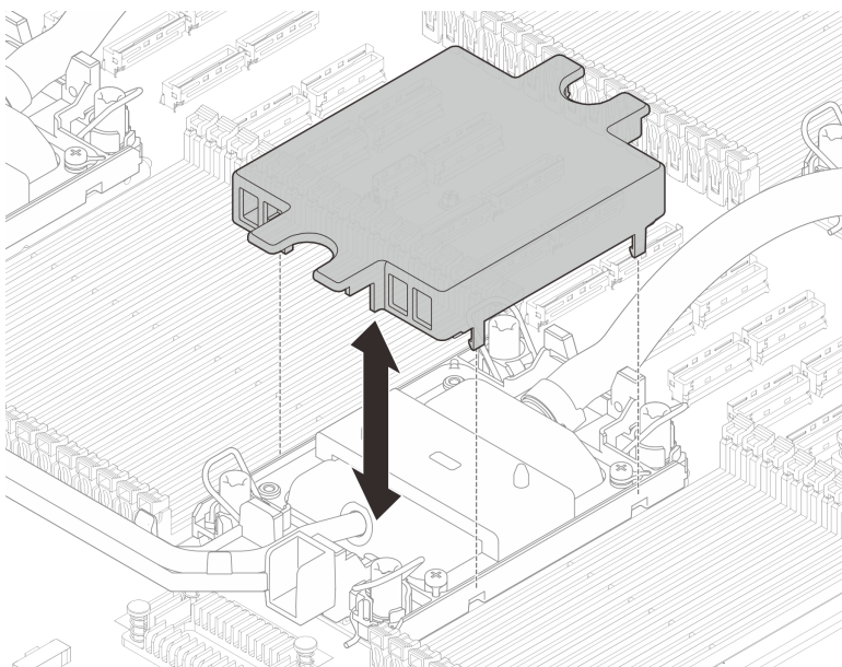
Рис. 93. Установка кожухов плат охлаждения
