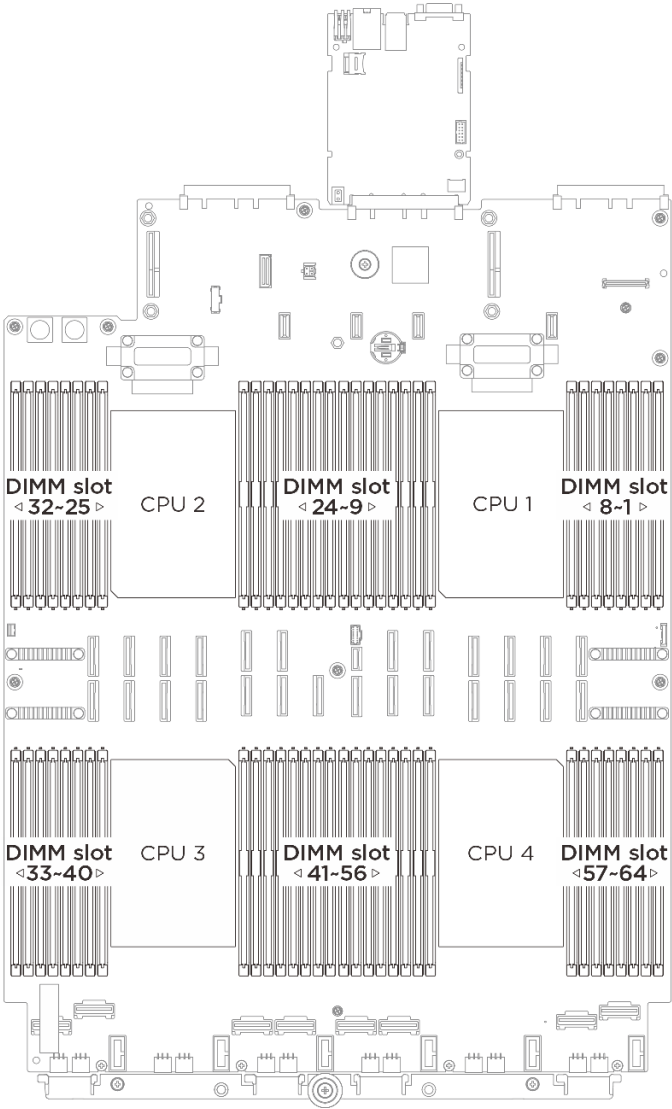
Рис. 1. Расположение модулей памяти и процессоров
