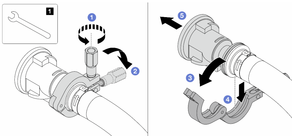
Рис. 120. Отделение шаровых клапанов
