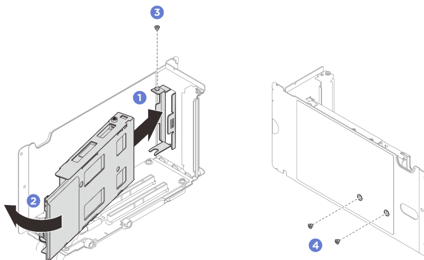
Рис. 210. Установка отсека для дисков M.2
