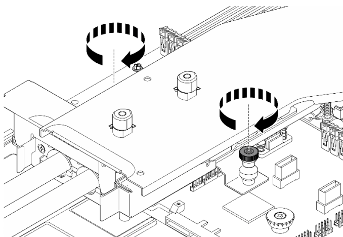
Рис. 89. Установка блока платы охлаждения
