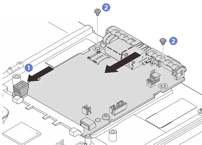
Рис. 226. Установка системной платы ввода-вывода
