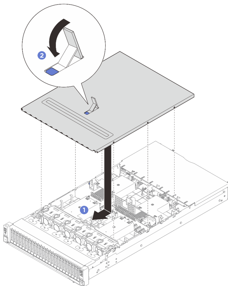
Рис. 236. Установка переднего верхнего кожуха
