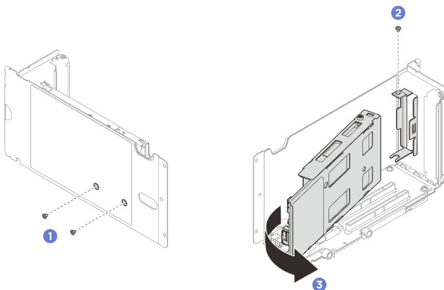
Рис. 207. Снятие отсека для дисков M.2
