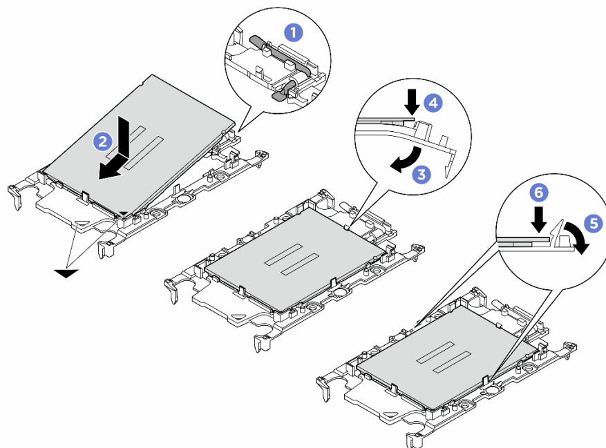
Рис. 196. Установка держателя процессора
