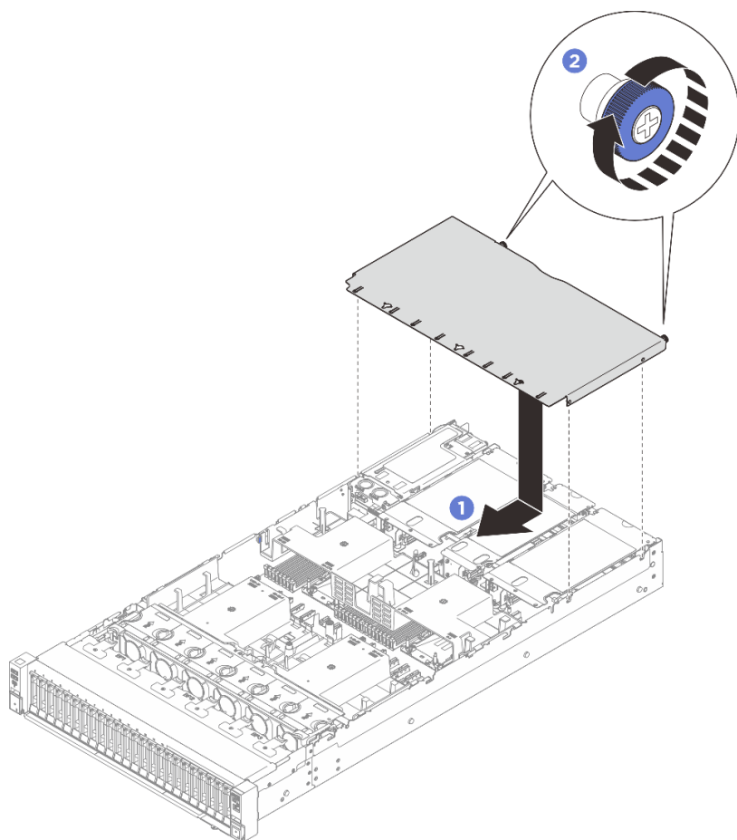
Рис. 235. Установка заднего верхнего кожуха
