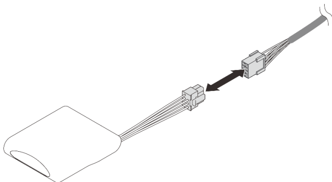
Рис. 19. Подключение кабеля модуля питания флэш-памяти
