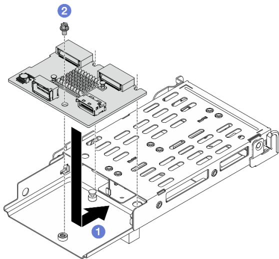
Рис. 209. Установка адаптера загрузки M.2
