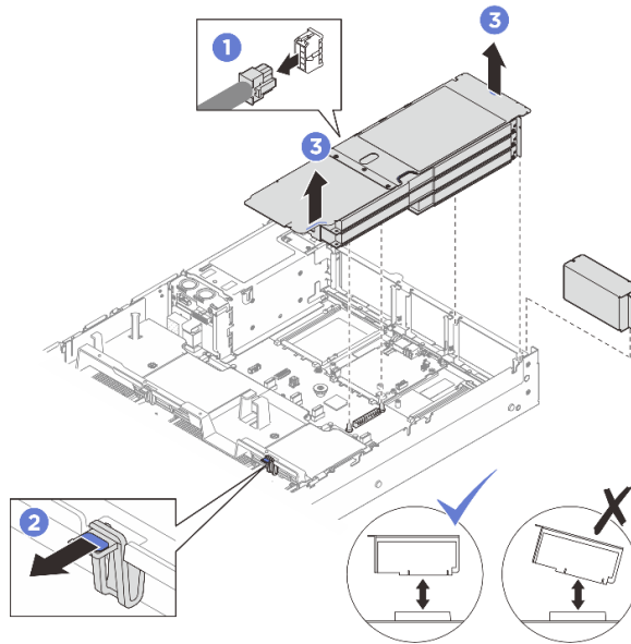
Рис. 165. Снятие платы-адаптера Riser PCIe максимальной высоты, полной длины
