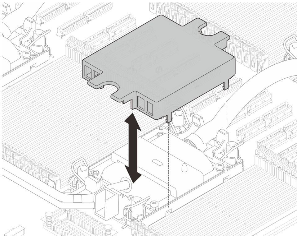
Рис. 258. Снятие кожуха платы охлаждения
