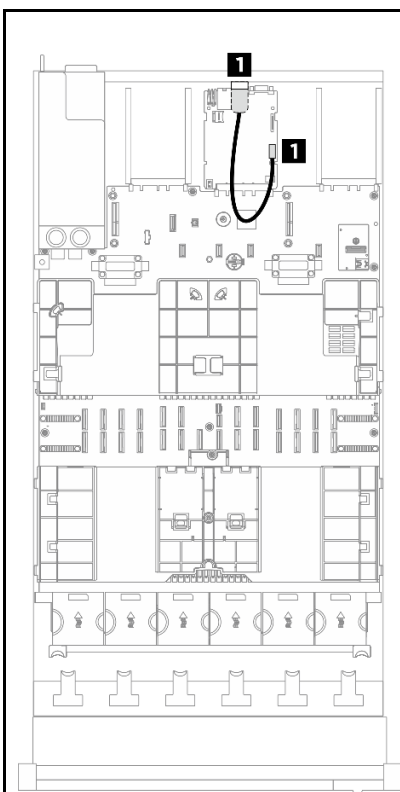
Рис. 221. Прокладка кабеля для модуля последовательного порта для модели сервера с тремя платами-адаптерами Riser PCIe
