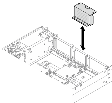
Рис. 94. Установка заглушки платы-адаптера Riser
