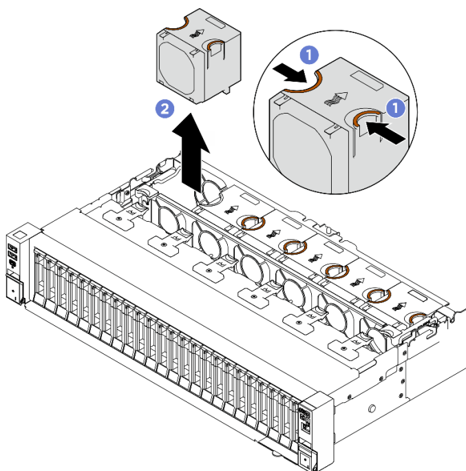
Рис. 49. Снятие вентилятора
