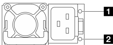
Рис. 248. Светодиодные индикаторы на модуле блока питания CRPS Premium (CFFv5)
