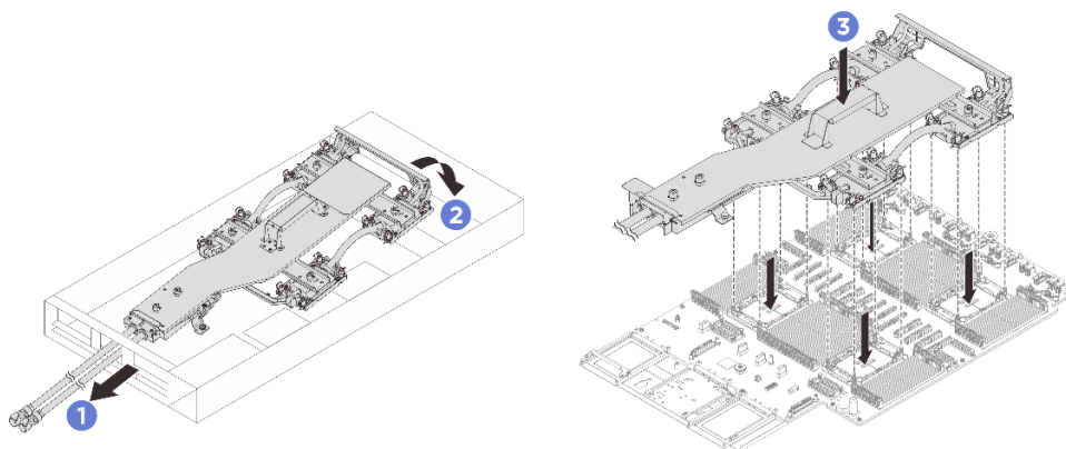
Рис. 88. Установка блока платы охлаждения
