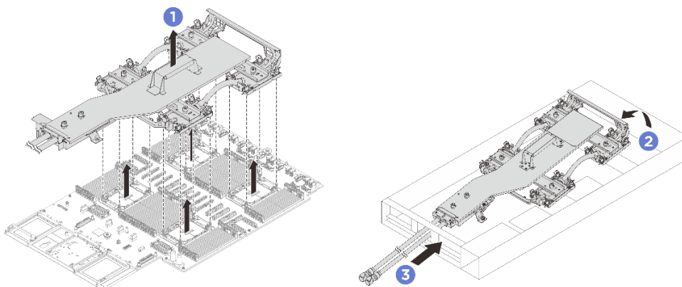
Рис. 84. Снятие блока платы охлаждения
