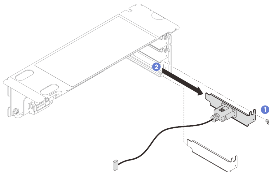
Рис. 218. Извлечение модуля последовательного порта
