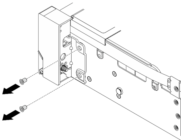
Рис. 202. Извлечение винтов
