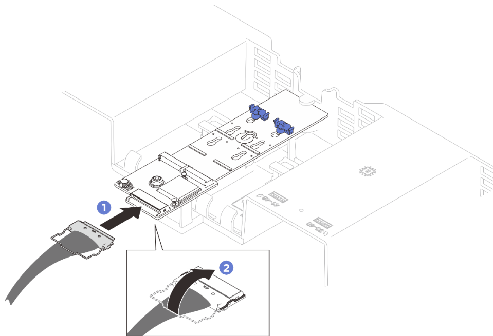
Рис. 100. Подключение кабелей адаптера загрузки M.2
