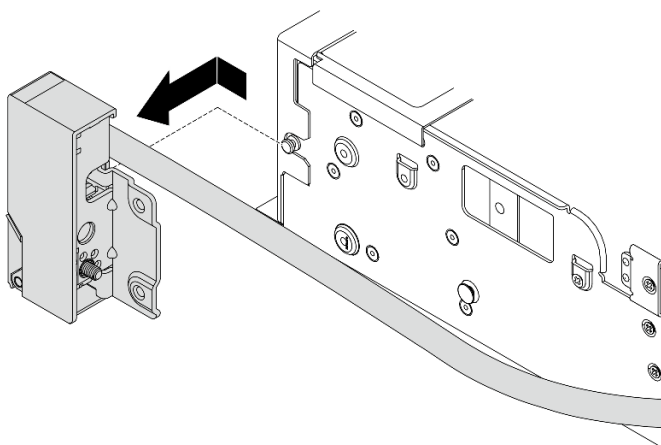
Рис. 203. Снятие защелки стойки
