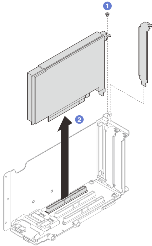
รูปภาพ 166. การถอดอะแดปเตอร์ PCIe
