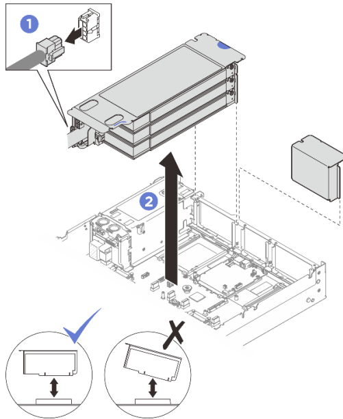
รูปภาพ 163. การถอดด้วยก PCIe LP (มีขั้วต่อไฟฟ้า)
