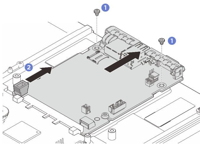
รูปภาพ 229. การถอดแผง I/O ระบบ
