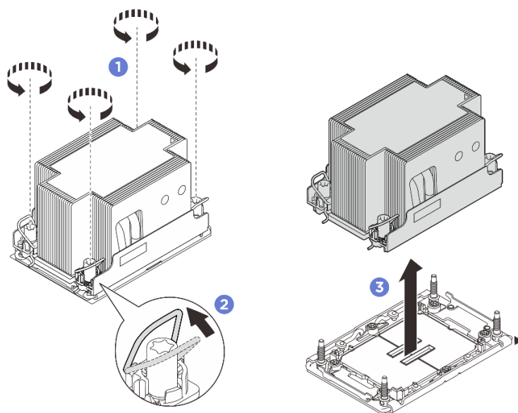
รูปภาพ 191. การถอด PHM แบบมาตรฐาน 2U
