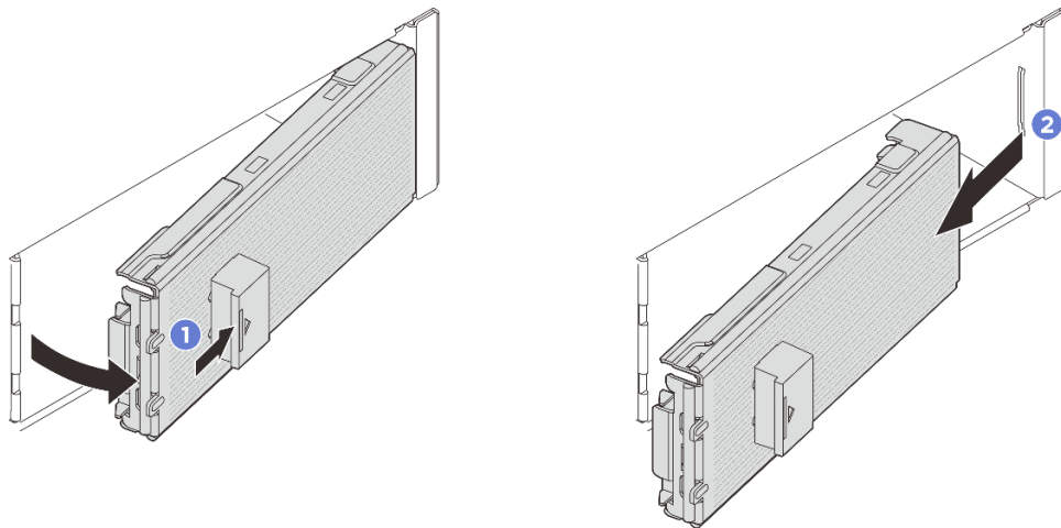
รูปภาพ 24. การถอดฝา E3.S
