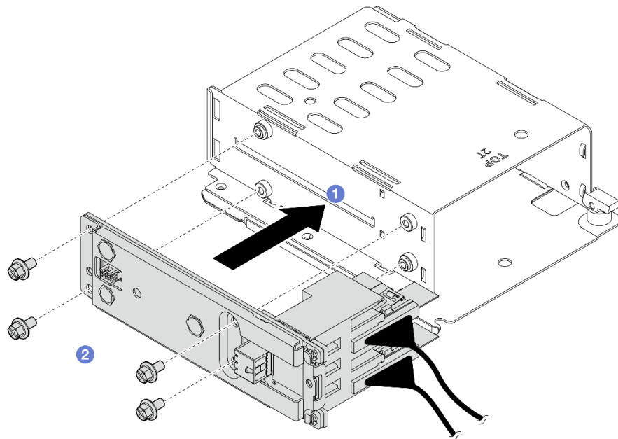
รูปภาพ 35. การติดตั้งแบ็คเพลน
