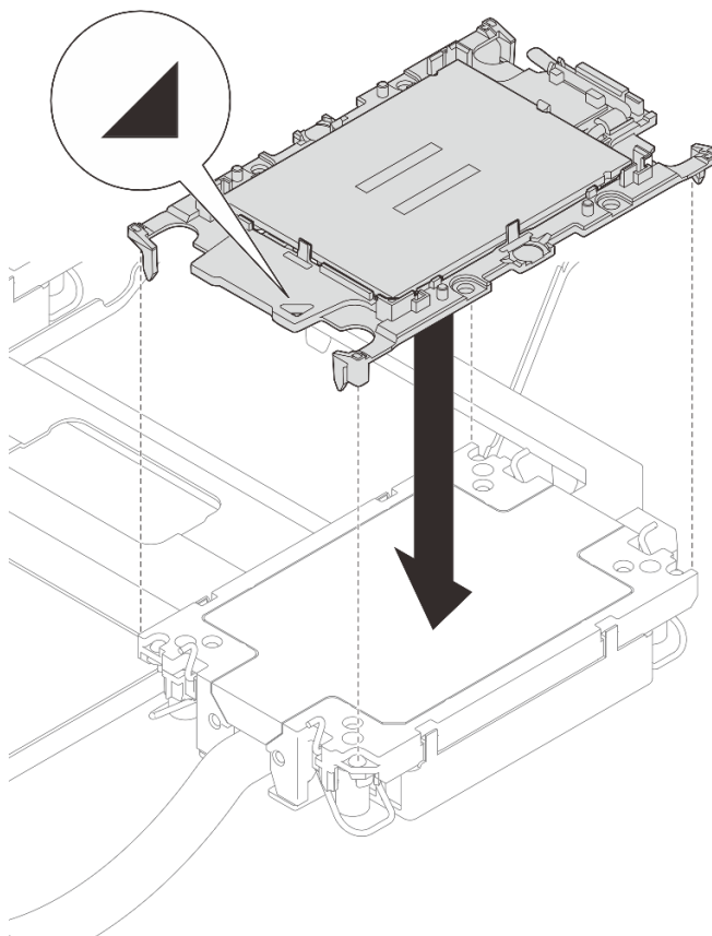
รูปภาพ 87. การติดตั้งโปรเซสเซอร์ลงในแผ่นระบายความร้อน
