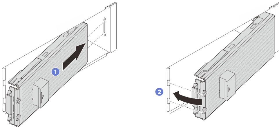
รูปภาพ 32. การติดตั้งฝา E3.S
