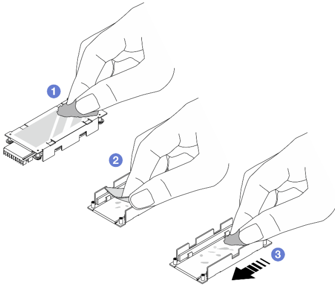
รูปภาพ 68. การทำความสะอาดแผ่นระบายความร้อนและแผ่นด้านล่าง
