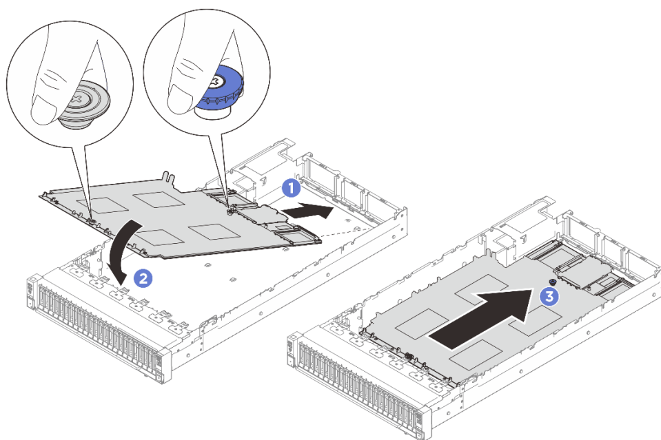
รูปภาพ 227. การติดตั้งส่วนประกอบแผงระบบ
