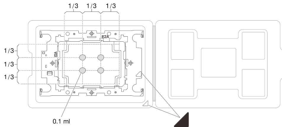
รูปภาพ 197. การทาครีมระบายความร้อนให้กับโปรเซสเซอร์ในภาคสำหรับจัดส่ง
