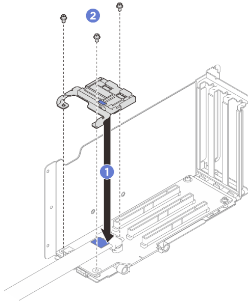
รูปภาพ 182. การติดตั้งตัวยึด PCIe
