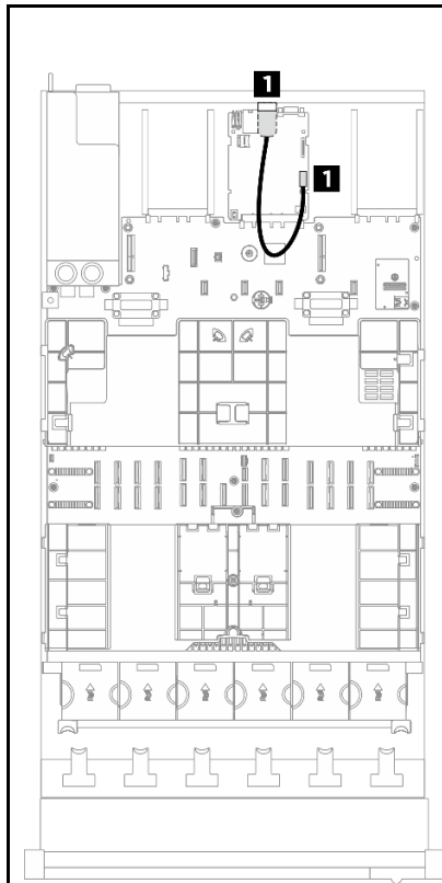
รูปภาพ 221. การเดินสายโมดูลพอร์ตอนุกรมสำหรับ รุ่นเซิร์ฟเวอร์ที่มีตัวยก PCIe สามตัว
