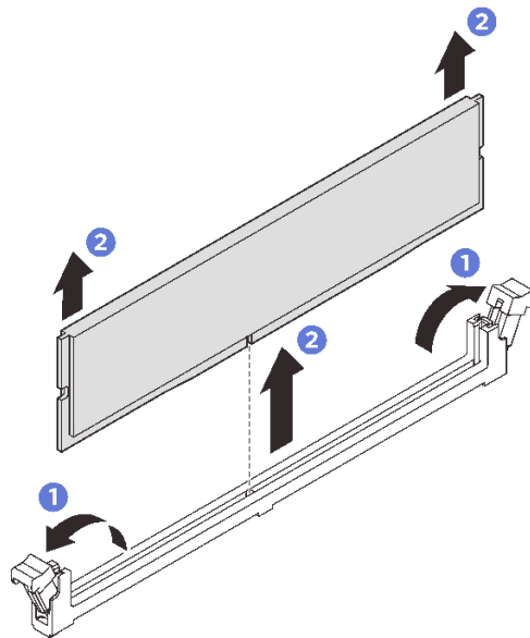
รูปภาพ 153. การถอดโมดูลหน่วยความจำ
