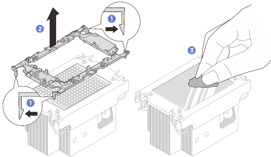
รูปภาพ 194. การแยกตัวนำโปรเซสเซอร์ออกจากตัวระบายความร้อน
