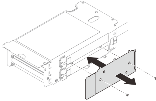
รูปภาพ 180. การติดตั้งฝาครอบสาย
