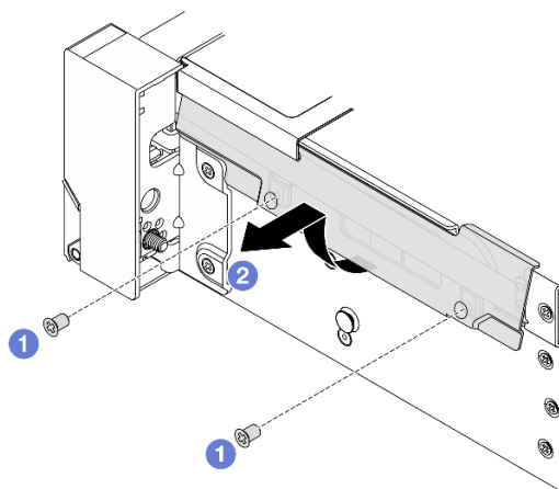
รูปภาพ 201. การถอดตัวยึดสาย
