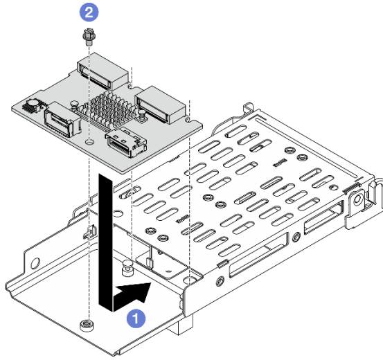
รูปภาพ 209. การติดตั้งอะแดปเตอร์ M.2
