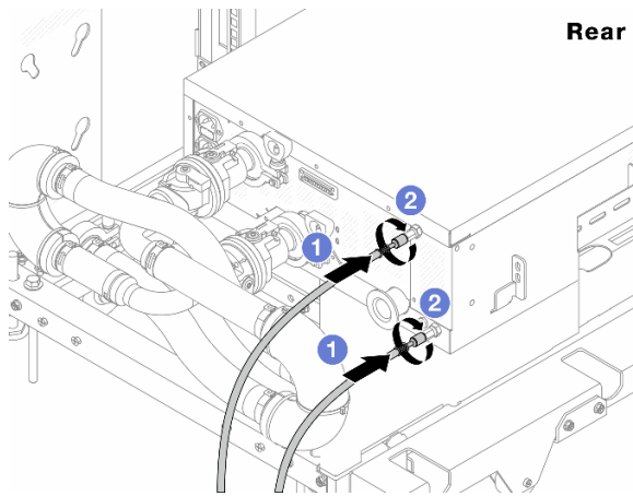
รูปภาพ 125. ด้านหลังของ CDU
