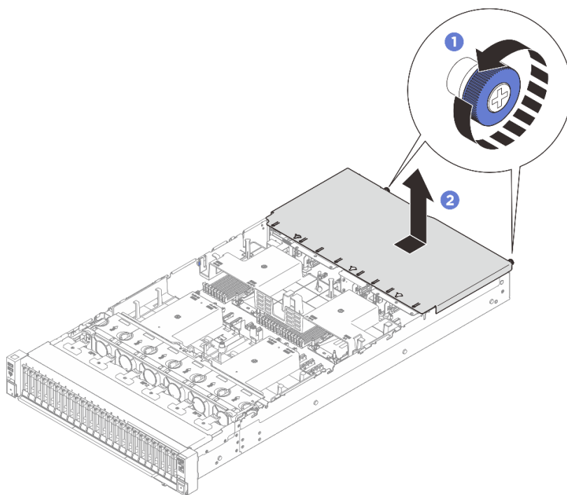
รูปภาพ 234. การถอดฝาครอบด้านบนด้านหลัง
