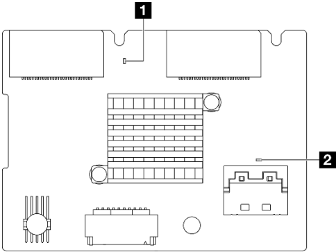
รูปภาพ 252. ไฟ LED อะแดปเตอร์บูต M.2 ด้านหลัง
