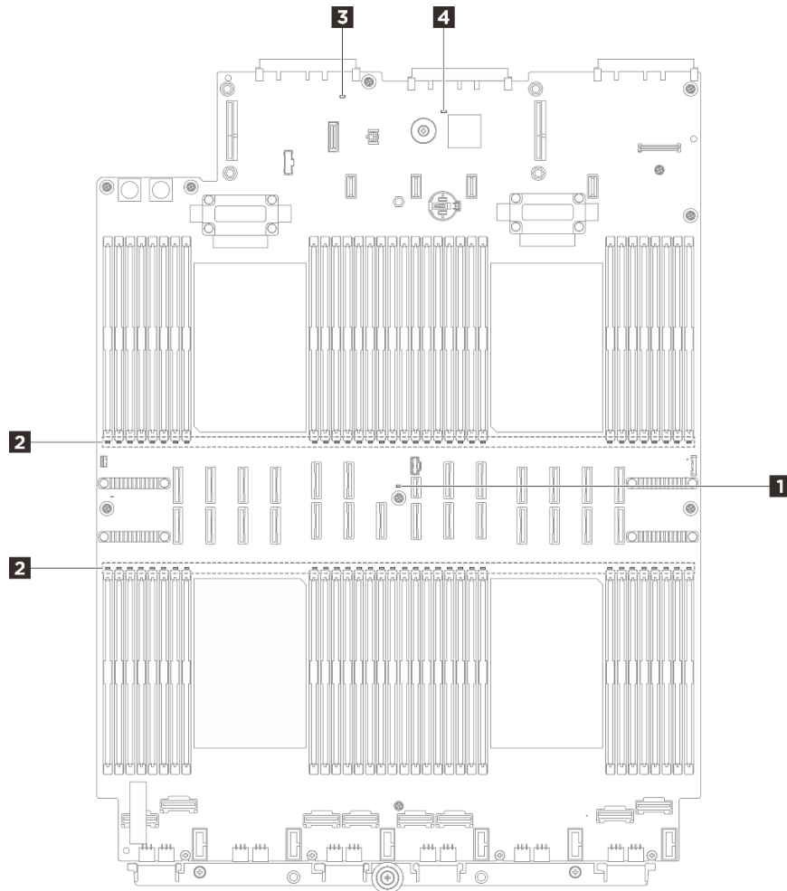
รูปภาพ 254. ไฟ LED บนแผงโปรเซสเซอร์
