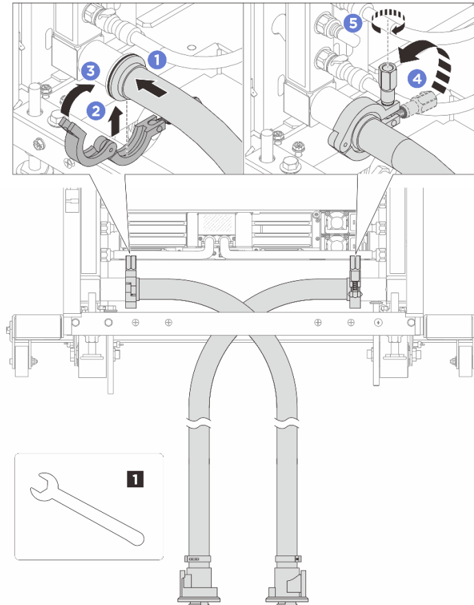
รูปภาพ 143. การติดตั้งชุดสาย
