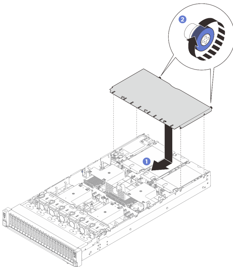
รูปภาพ 235. การติดตั้งฝาครอบด้านบนด้านหลัง
