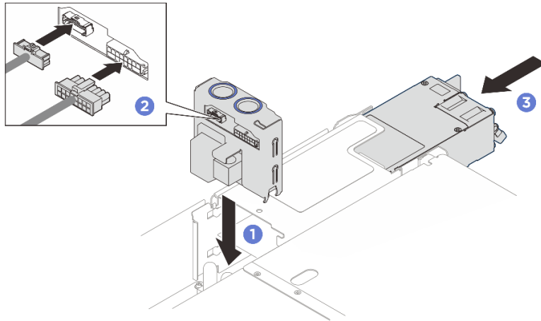
รูปภาพ 187. การติดตั้งแผงจ่ายไฟ
