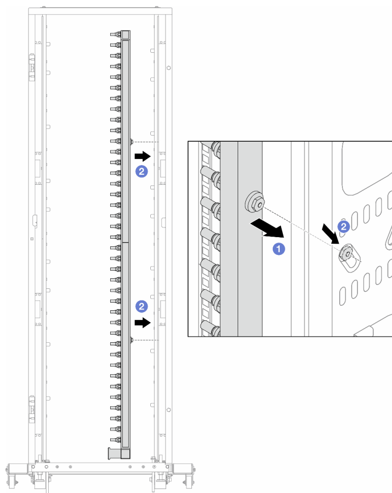
รูปภาพ 141. การติดตั้งท่อ
