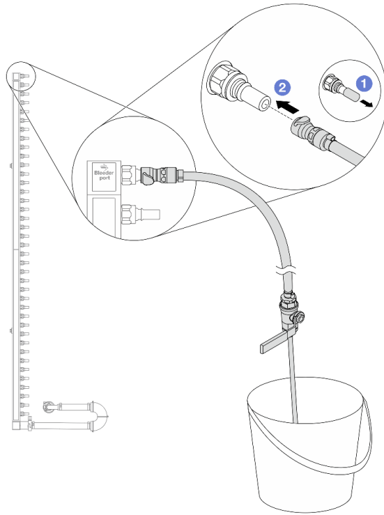
รูปภาพ 114. การติดตั้งชุดวาล์วหรือเข้ากับฝั่งจ่าย
