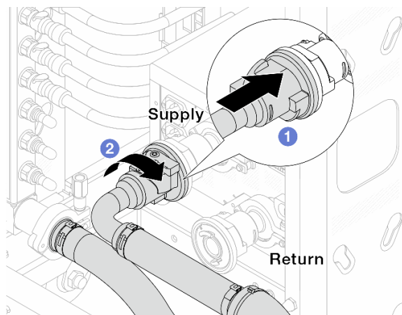
รูปภาพ 123. การเชื่อมต่อบอลวาล์ว
