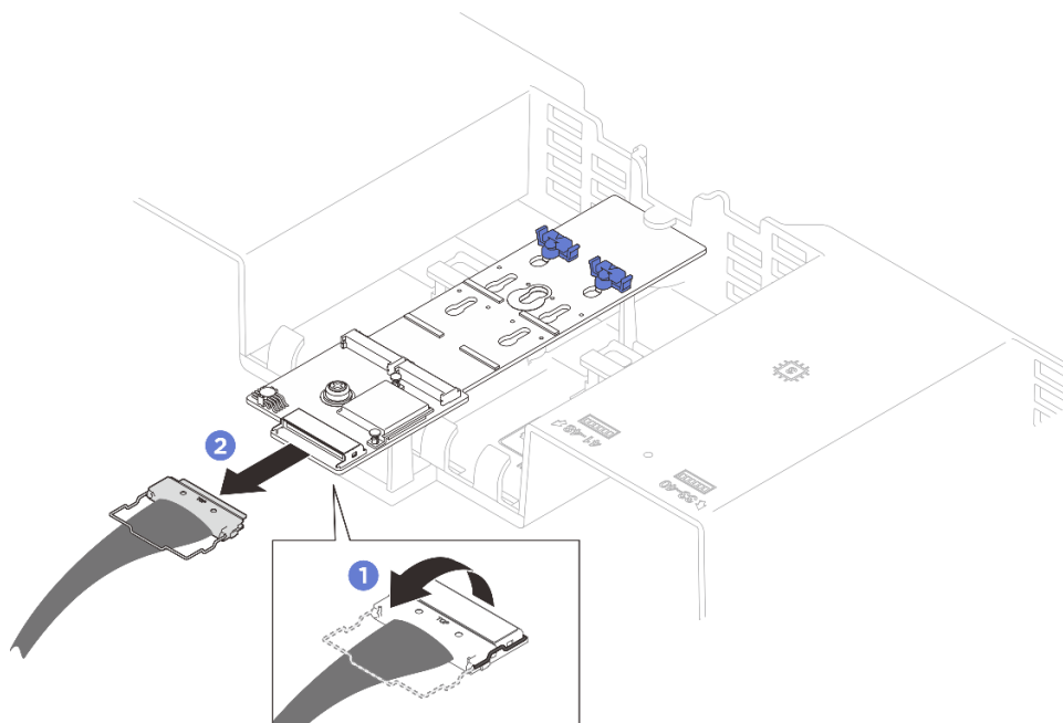
รูปภาพ 9. การถอดสายอะแดปเตอร์ M.2
