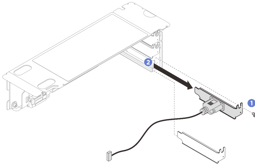
รูปภาพ 218. การถอดโมดูลพอร์ตอนุกรม
