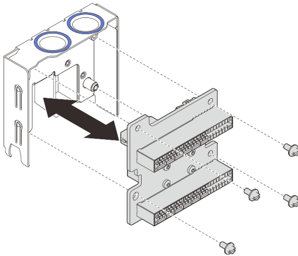
รูปภาพ 186. การแยกชิ้นส่วนของแผงจ่ายไฟ
