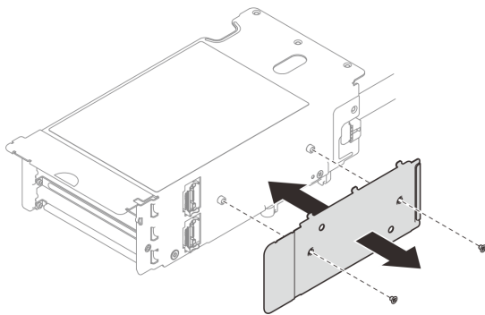
รูปภาพ 177. การถอดฝาครอบสาย
