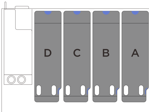
รูปภาพ 162. รูนเซิร์ฟเวอร์ที่มีตัวยก PCIe สี่ตัว
