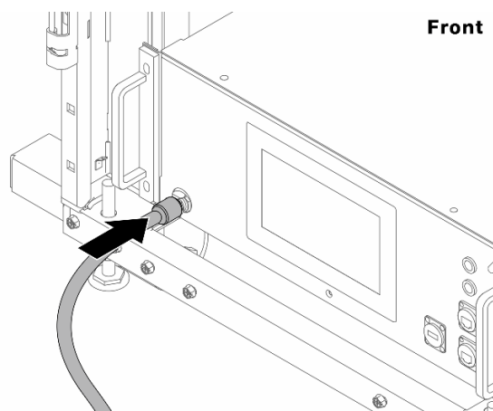
รูปภาพ 124. ด้านหน้าของ CDU
