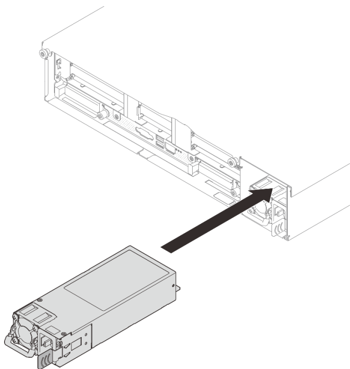
รูปภาพ 189. การติดตั้งชุดแหล่งจ่ายไฟ
