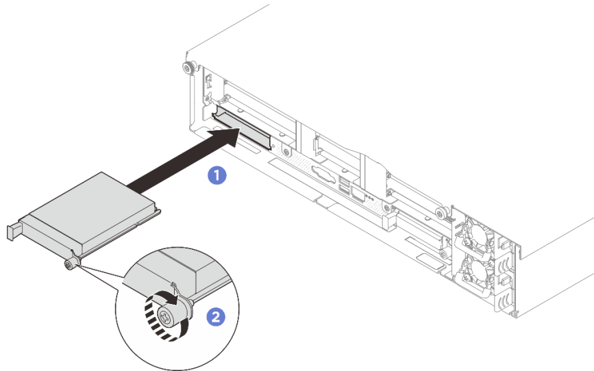
รูปภาพ 159. การติดตั้งโมดูล OCP
