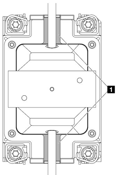
รูปภาพ 257. พื้นที่ที่อาจเกิดการรั่วไหล
