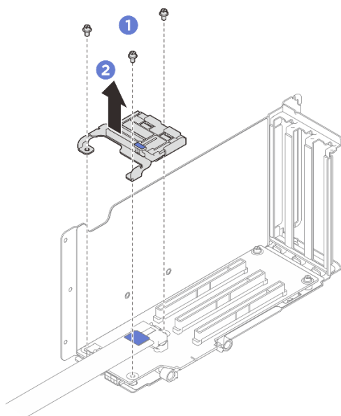
รูปภาพ 181. การถอดตัวยึด PCIe
