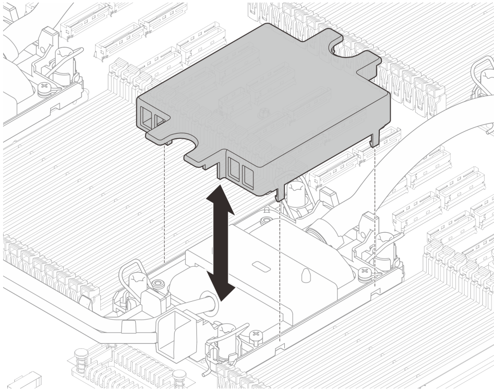
รูปภาพ 258. การถอดฝาครอบแผ่นระบายความร้อน
