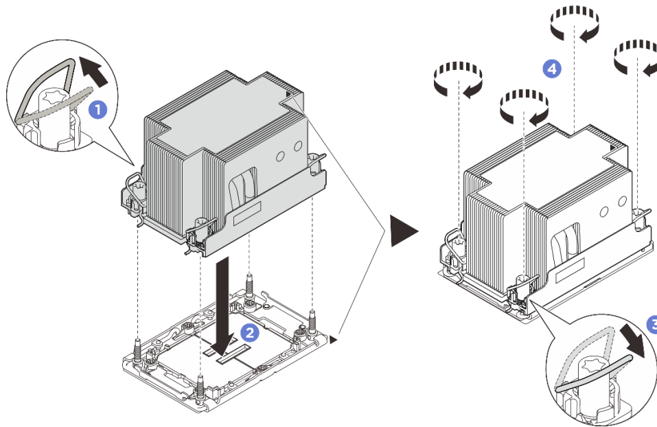
รูปภาพ 199. การติดตั้ง PHM แบบมาตรฐาน 2U
