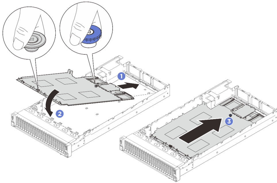
รูปภาพ 231. การติดตั้งส่วนประกอบแผงระบบ
