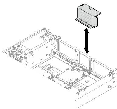
รูปภาพ 94. การติดตั้งแผงครอบตัวยก
