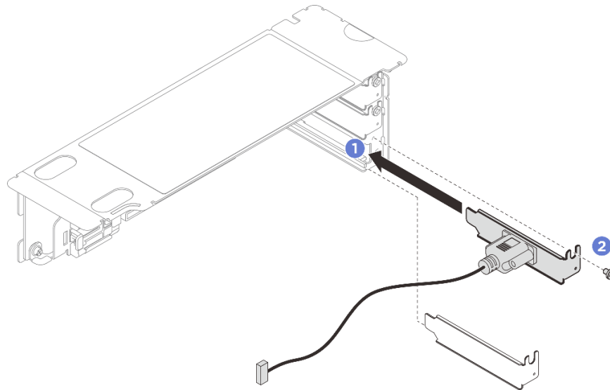
รูปภาพ 219. การติดตั้งโมดูลพอร์ตอนุกรม
