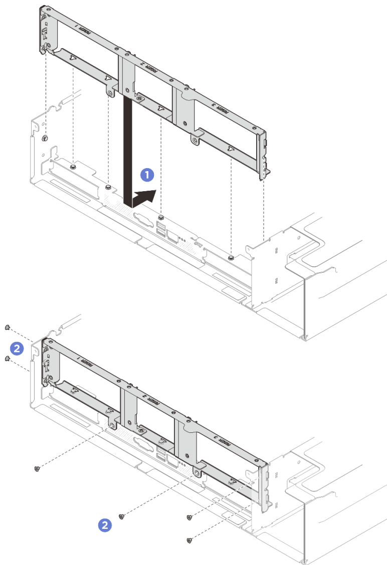
รูปภาพ 212. การติดตั้งผนังด้านหลัง
