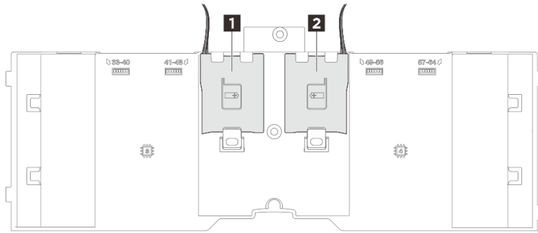
รูปภาพ 55. ตำแหน่งช่องเสียบโมดูลพลังงานแบบแฟลช
