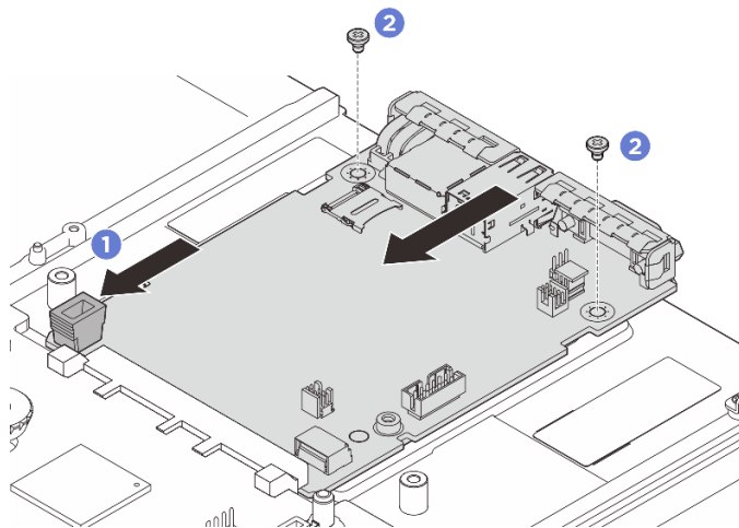
รูปภาพ 230. การติดตั้งแผง I/O ระบบ
