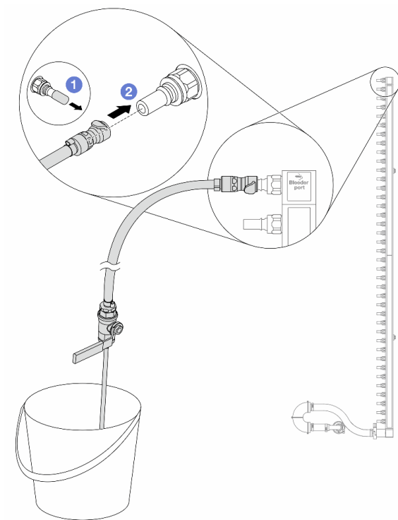
รูปภาพ 116. การติดตั้งชุดวาล์วหรือเข้ากับฝั่งหมุนเวียน
