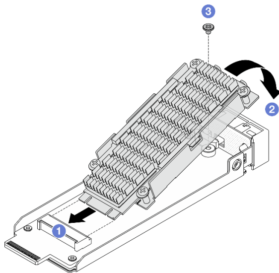
รูปภาพ 72. การติดตั้งไดรฟ์ M.2 พร้อมตัวระบายความร้อน
