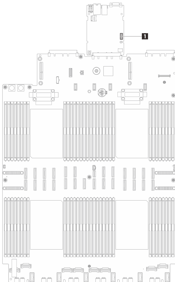
รูปภาพ 220. ตำแหน่งของหัวต่อพอร์ตอนุกรม
