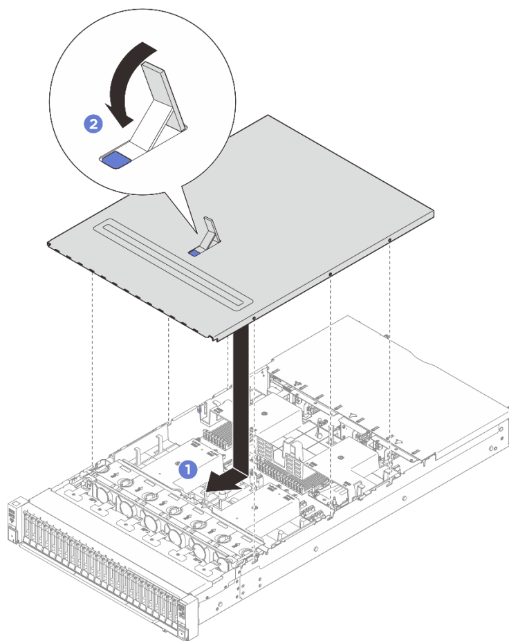
รูปภาพ 236. การติดตั้งฝาครอบด้านหน้าด้านบน
