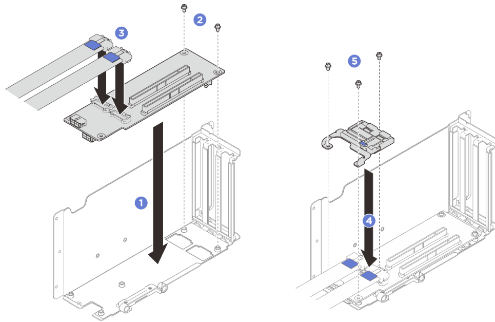
รูปภาพ 178. การติดตั้งการ์ดด้วยก PCIe
