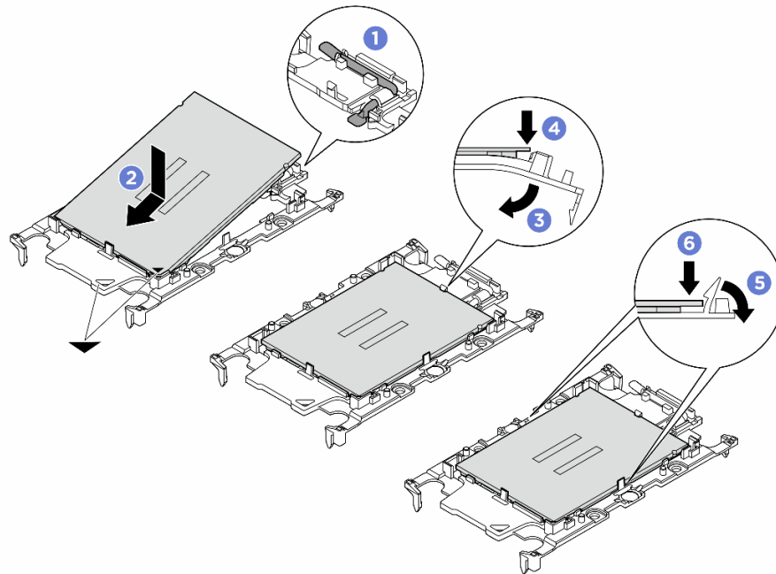
รูปภาพ 196. การติดตั้งตัวนำโปรเซสเซอร์
