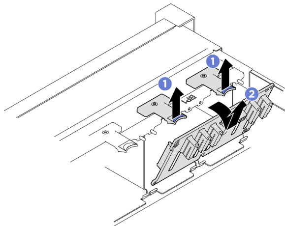
รูปภาพ 5. การถอดไดรฟ์แบ็คเพลนขนาด 2.5 นิ้ว
