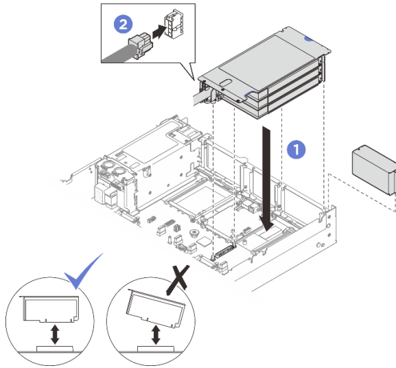
รูปภาพ 172. การติดตั้งตัวยก PCIe FHHL
