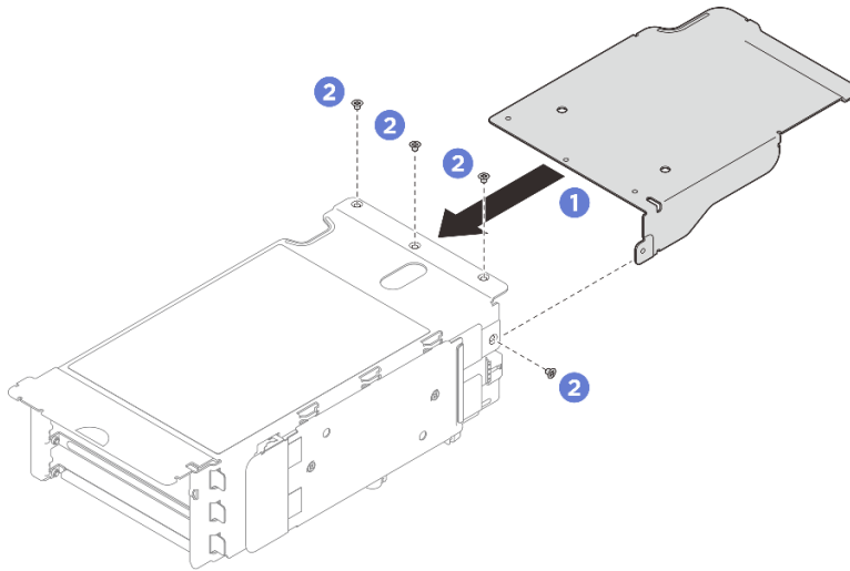
รูปภาพ 184. การติดตั้งตัวขยายตัวยก PCIe
