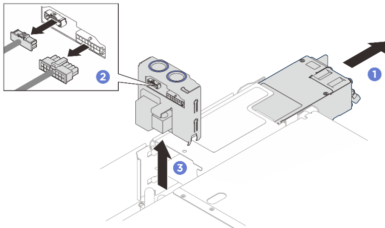
รูปภาพ 185. การถอดแผงจ่ายไฟ
