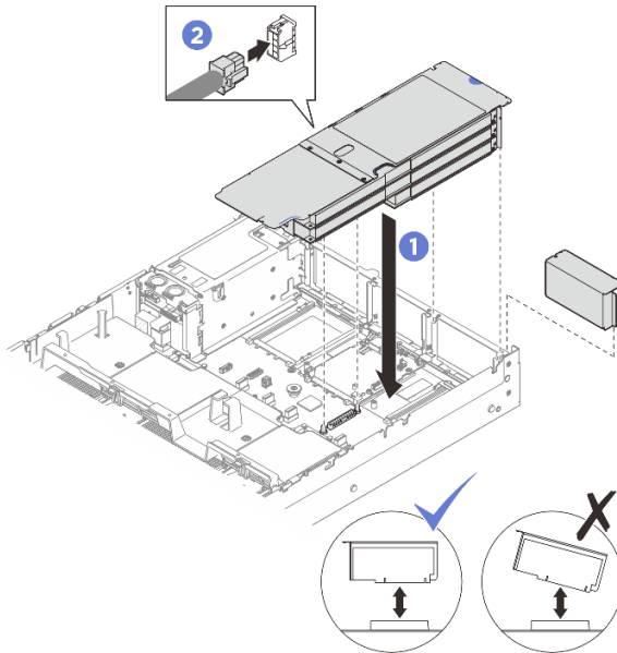
รูปภาพ 173. การติดตั้งตัวยก PCIe FHFL
