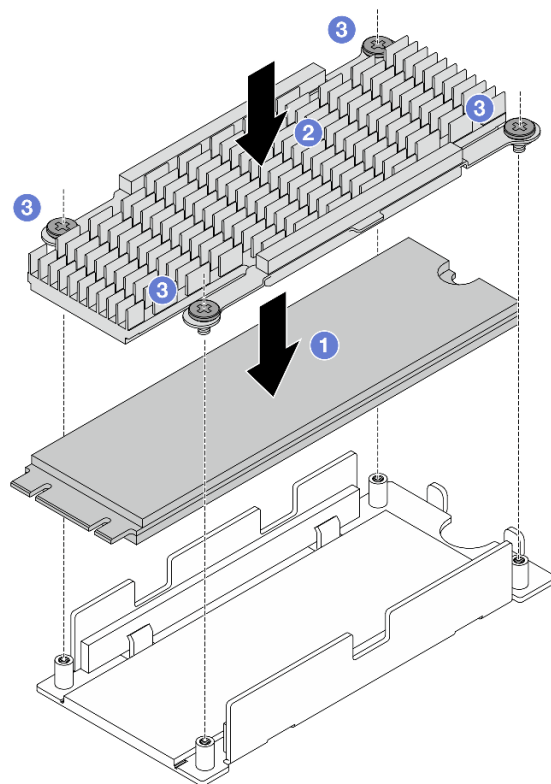
รูปภาพ 70. การประกอบตัวระบายความร้อนและไดรฟ์ M.2
