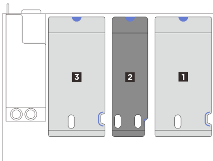
รูปภาพ 160. รูนเซิร์ฟเวอร์ที่มีตัวยก PCIe สามตัว
