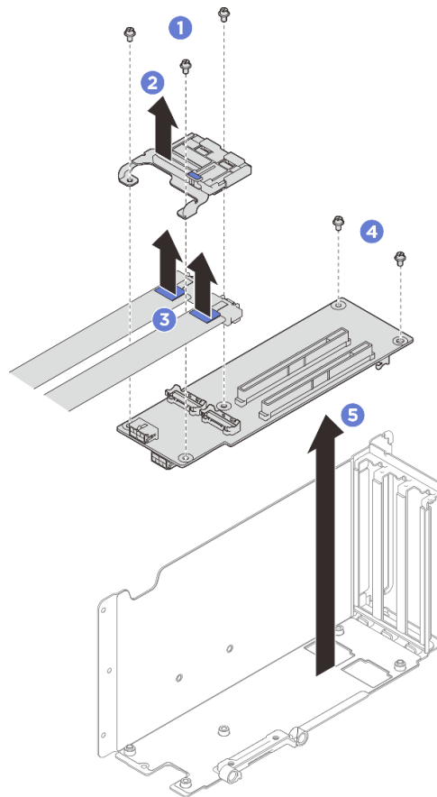
รูปภาพ 176. การถอดการ์ดด้วยก PCIe
