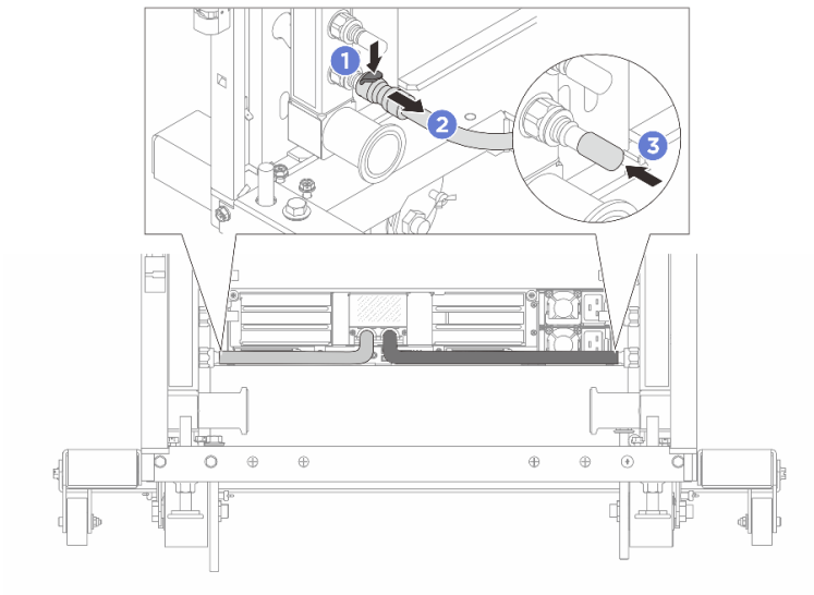
รูปภาพ 134. การถอดปลั๊ก Quick Connect
