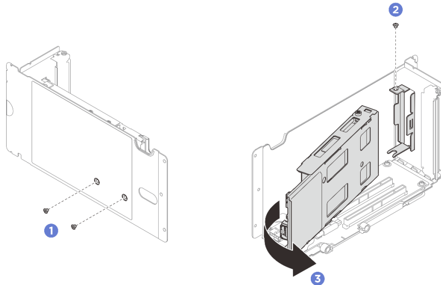
รูปภาพ 207. การถอดตัวครอบไดรฟ์ M.2
