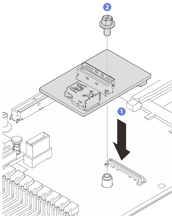
รูปภาพ 239. การติดตั้งแผง I/O USB
