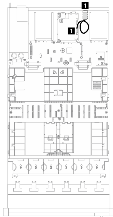
รูปภาพ 222. การเดินสายโมดูลพอร์ตอนุกรมสำหรับ รุ่นเซิร์ฟเวอร์ที่มีตัวยก PCIe สี่ตัว
