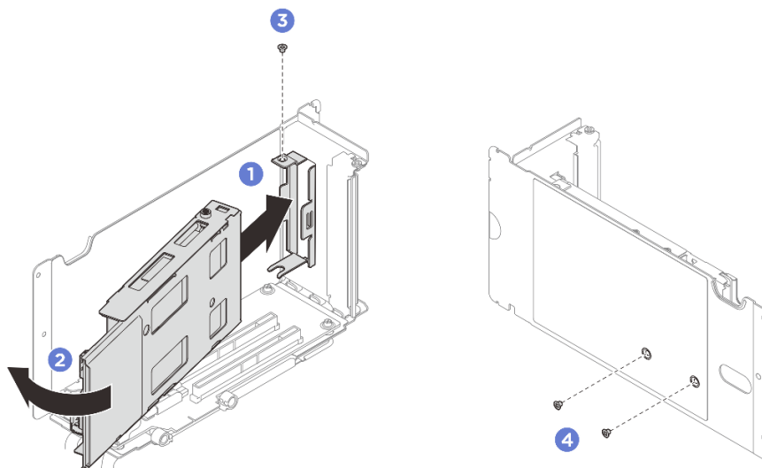
รูปภาพ 210. การติดตั้งตัวครอบไดรฟ์ M.2
