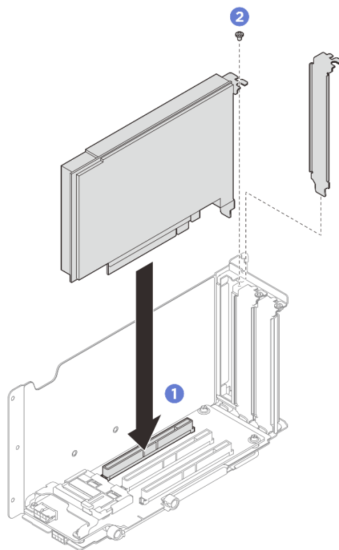
รูปภาพ 167. การติดตั้งอะแดปเตอร์ PCIe
