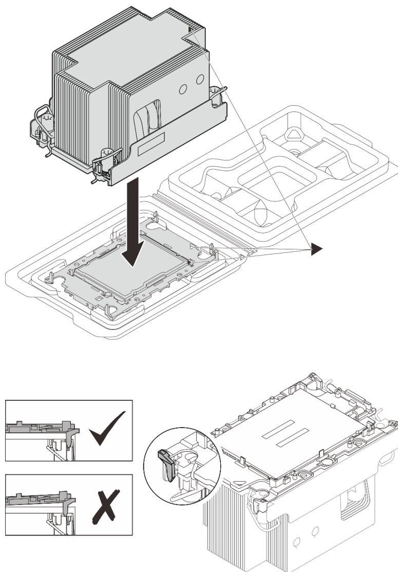
รูปภาพ 198. การประกอบ PHM พร้อมโปรเซสเซอร์ในถาดสำหรับจัดส่ง
