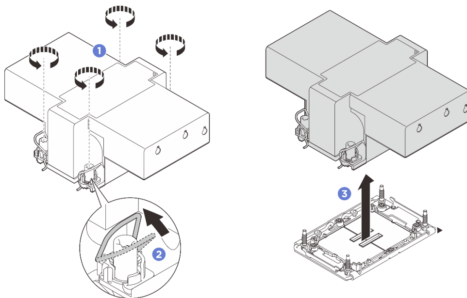
รูปภาพ 192. การถอด PHM แบบประสิทธิภาพสูง 2U
