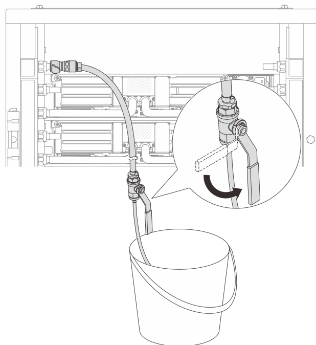
รูปภาพ 150. การเปิดวาล์วหรือบนฝั่งจ่าย
