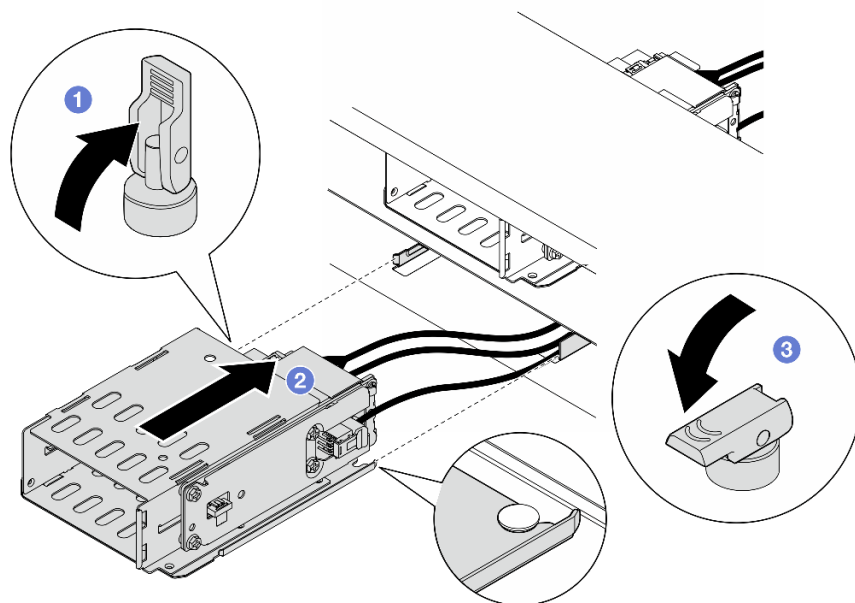
รูปภาพ 36. การติดตั้งตัวครอบ E3.S 2T
