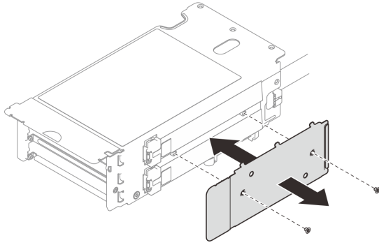
รูปภาพ 174. การถอดฝาครอบสาย
