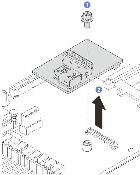
รูปภาพ 238. การถอดแผง I/O USB
