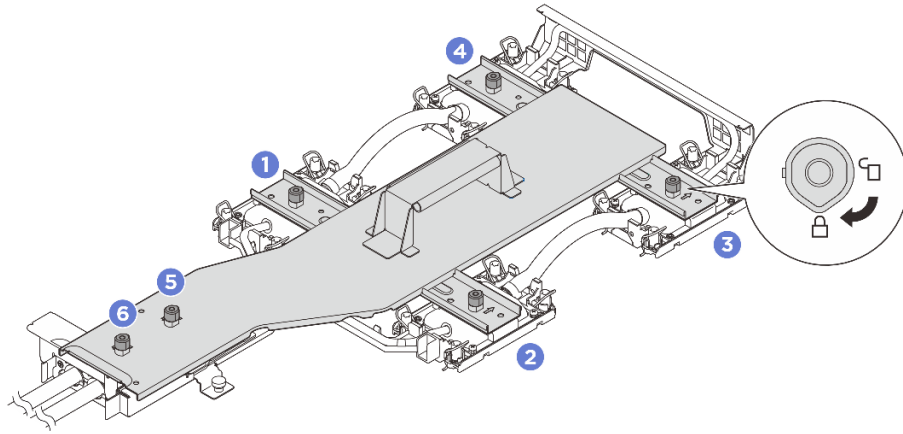
รูปภาพ 81. การยึดตัวยึดแผ่นระบายความร้อน
