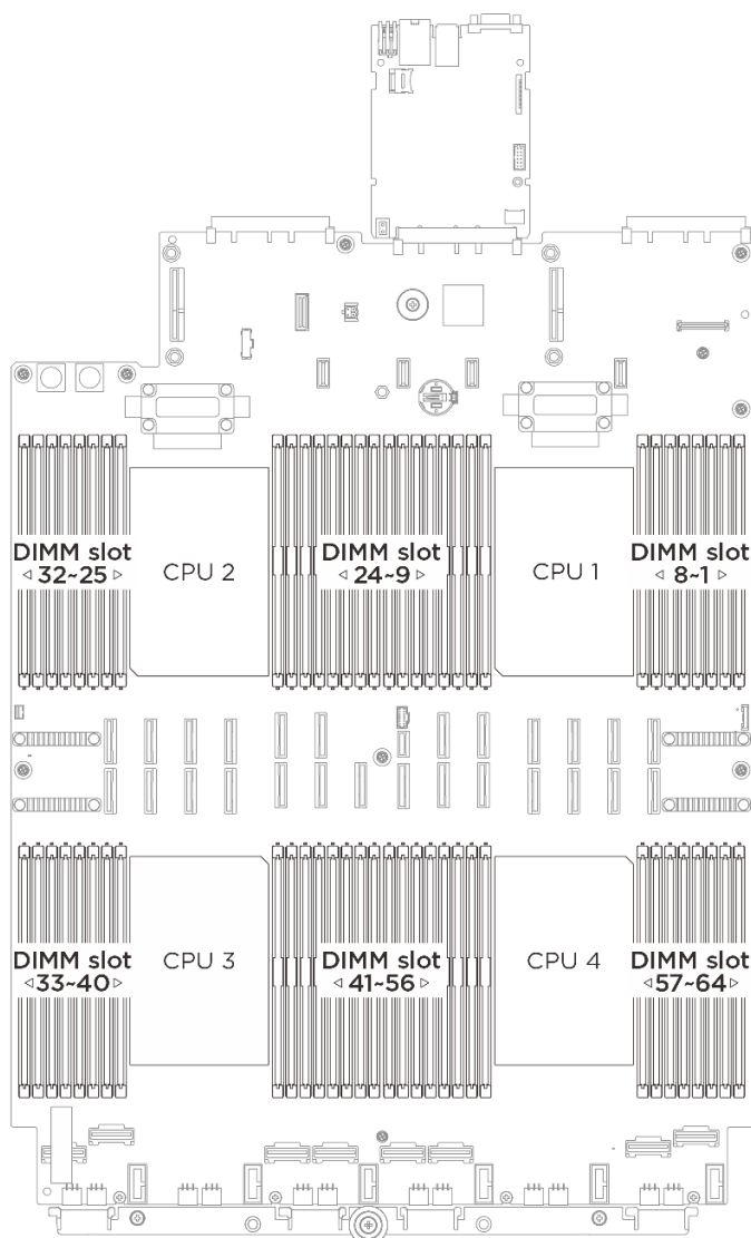
รูปภาพ 152. เค้าโครงโมดูลหน่วยความจำและโปรเซสเซอร์
