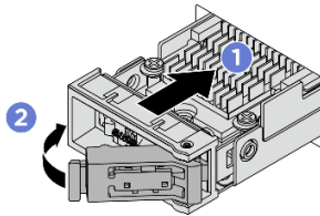
รูปภาพ 74. การติดตั้งส่วนประกอบไดรฟ์ M.2
