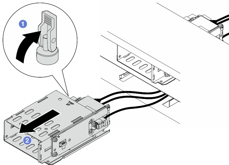
รูปภาพ 33. การถอดตัวครอบ E3.S 2T
