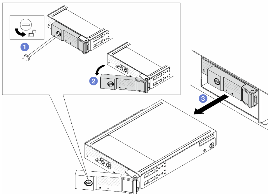
รูปภาพ 25. การถอด CMM
