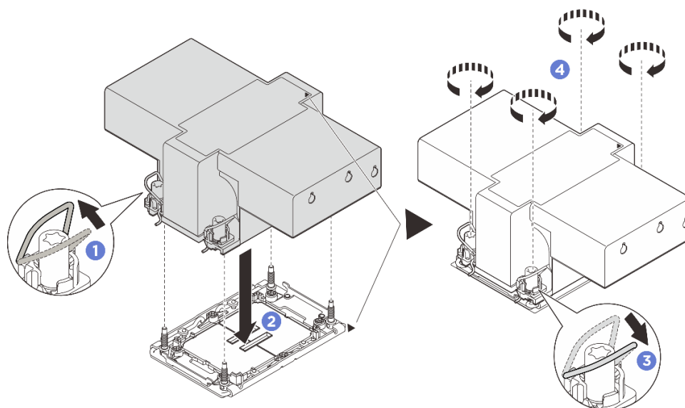
รูปภาพ 200. การติดตั้ง PHM แบบประสิทธิภาพสูง 2U
