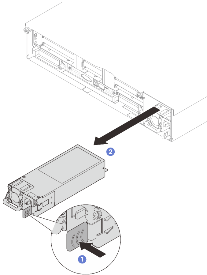
รูปภาพ 188. การถอดอุปกรณ์แหล่งพลังงาน
