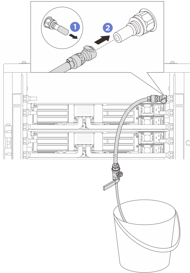
รูปภาพ 130. การติดตั้งชุดวาล์วหรือบนฝั้งหมุนเวียน
