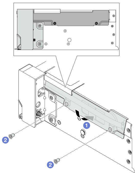
รูปภาพ 206. การติดตั้งตัวยึดสาย
