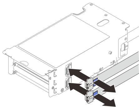
รูปภาพ 179. การเชื่อมต่อสาย
