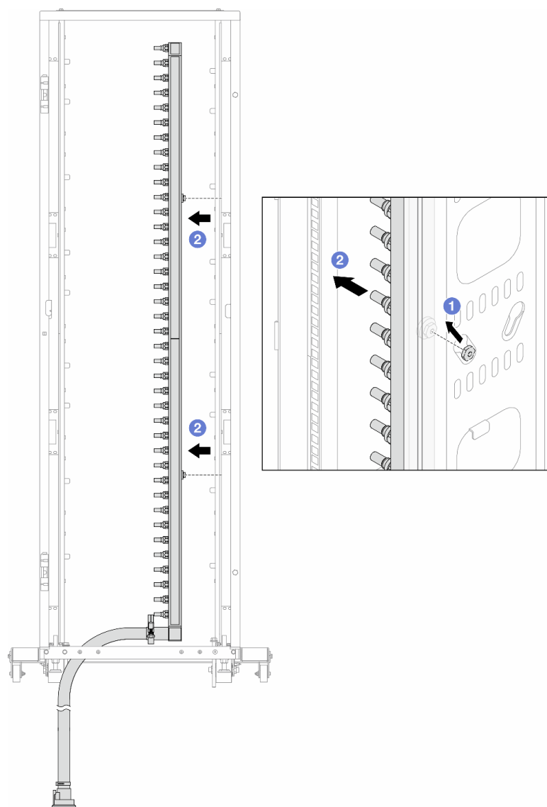
รูปภาพ 135. การถอดท่อ
