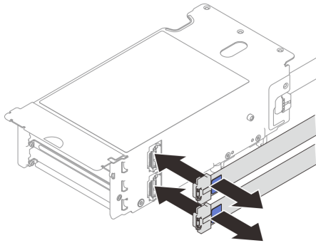
รูปภาพ 175. การถอดสายเคเบิล
