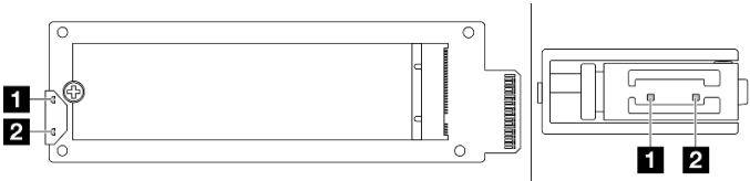
รูปภาพ 251. ไฟ LED อินเทอร์โพเซอร์ M.2 ด้านหลัง
