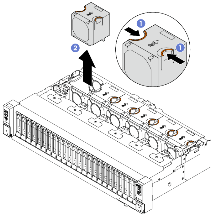
รูปภาพ 49. การถอดพัดลม
