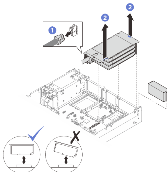
รูปภาพ 164. การถอดด้วยก PCIe FHHL
