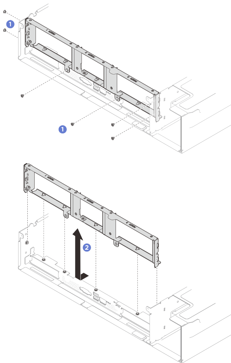
รูปภาพ 211. การถอดผนังด้านหลัง
