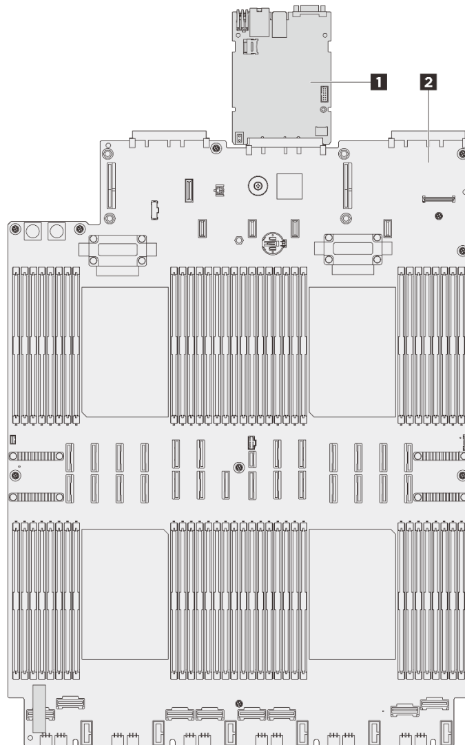
รูปภาพ 223. เค้าโครงส่วนประกอบแผงระบบ
