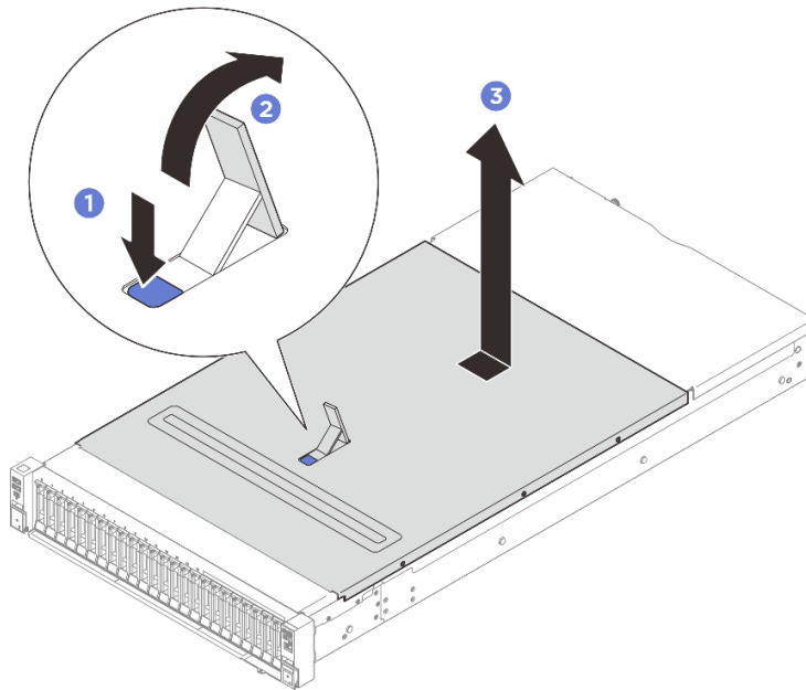
รูปภาพ 233. การถอดฝาครอบด้านบนด้านหน้า
