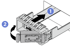
รูปภาพ 64. การติดตั้งถาดไดรฟ์ M.2
