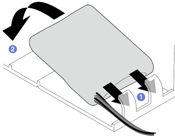
รูปภาพ 56. การติดตั้งโมดูลพลังงานแบบแฟลช
