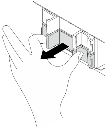
รูปภาพ 28. การถอดแผงครอบช่องใส่
