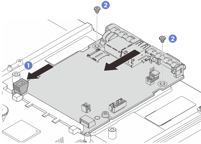
รูปภาพ 226. การติดตั้งแผง I/O ระบบ
