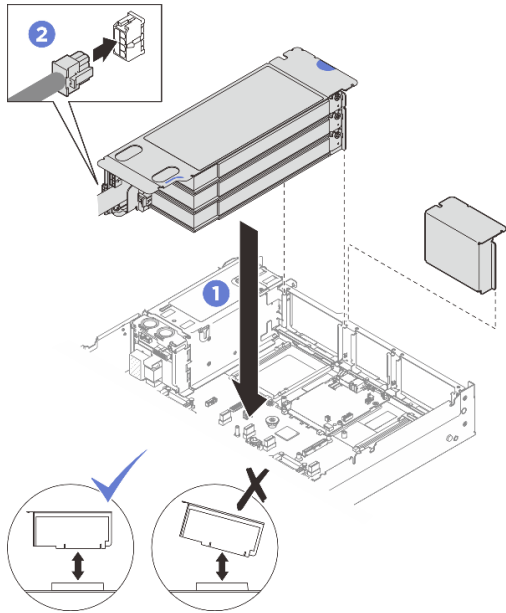
รูปภาพ 171. การติดตั้งตัวยก PCIe LP (มีหัวต่อไฟฟ้า)
