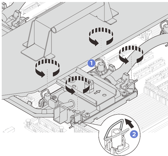
รูปภาพ 82. การคลายน็อต Torx T30
