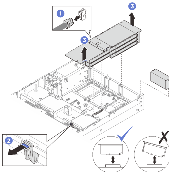
รูปภาพ 165. การถอดด้วยก PCIe FHFL
