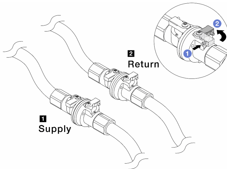
รูปภาพ 133. การปิดบอลวาล์ว
