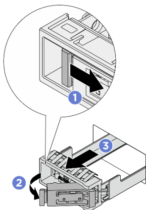
รูปภาพ 73. การถอดถาดไดรฟ์ M.2
