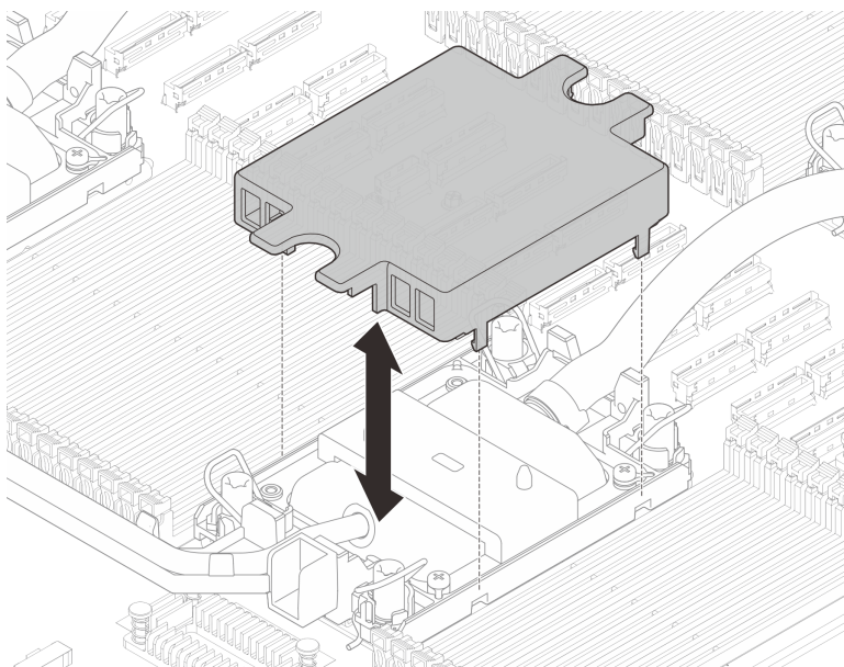
รูปภาพ 93. การติดตั้งแผ่นระบายความร้อน
