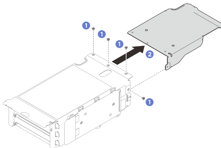
รูปภาพ 183. การถอดตัวย้ายด้วยก PCIe
