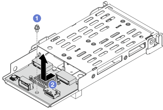
รูปภาพ 208. การถอดอะแดปเตอร์ M.2
