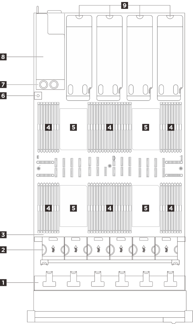
图 12. 配备四个 PCIe 转接卡的服务器型号的俯视图
