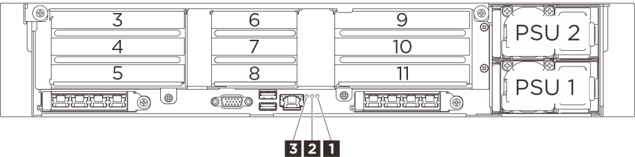
图 26. 背面系统 LED
