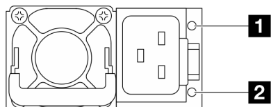
图 21. CRPS Premium（CFFv5）电源模块单元上的 LED
