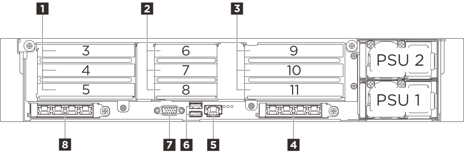
图 5. 配备三个 PCIe 转接卡的服务器型号的后视图
