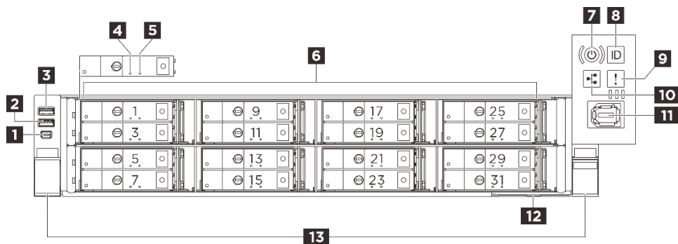
图 4. 配备 E3.S 2 T 插槽的服务器型号的前视图
