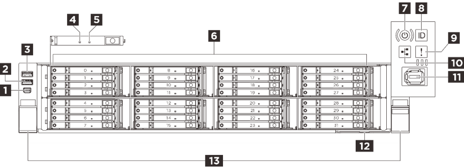
图 3. 配备 E3.S 1 T 插槽的服务器型号的前视图
