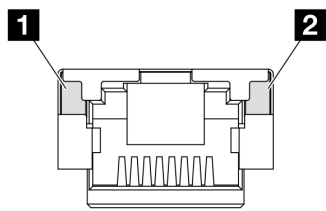
图 29. XCC 系统管理端口（10/100/1000 Mbps RJ-45）上的 LED
