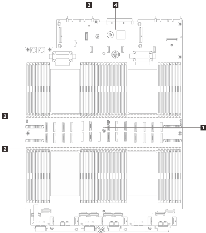
图 27. 处理器板 LED
