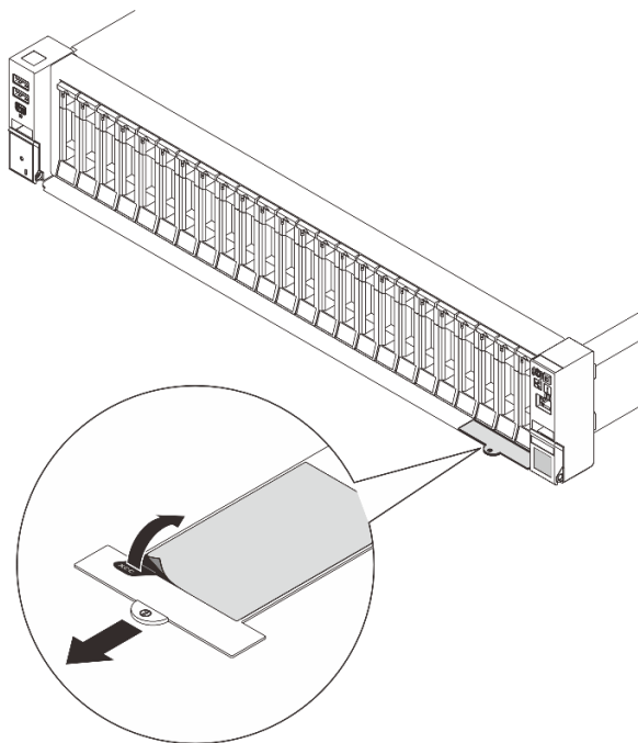
图 32. 抽取式信息卡上的 Lenovo XClarity Controller 网络访问标签
