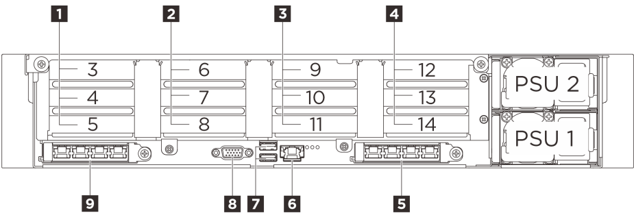
图 8. 配备四个 PCIe 转接卡的服务器型号的后视图
