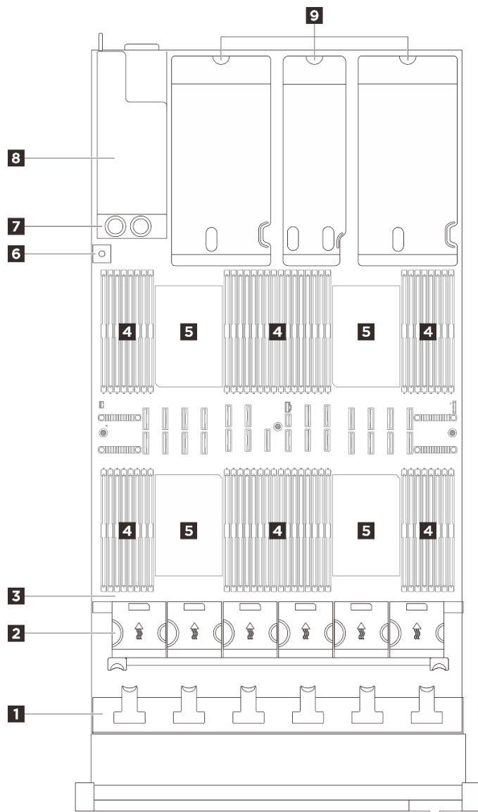
图 11. 配备三个 PCIe 转接卡的服务器型号的俯视图
