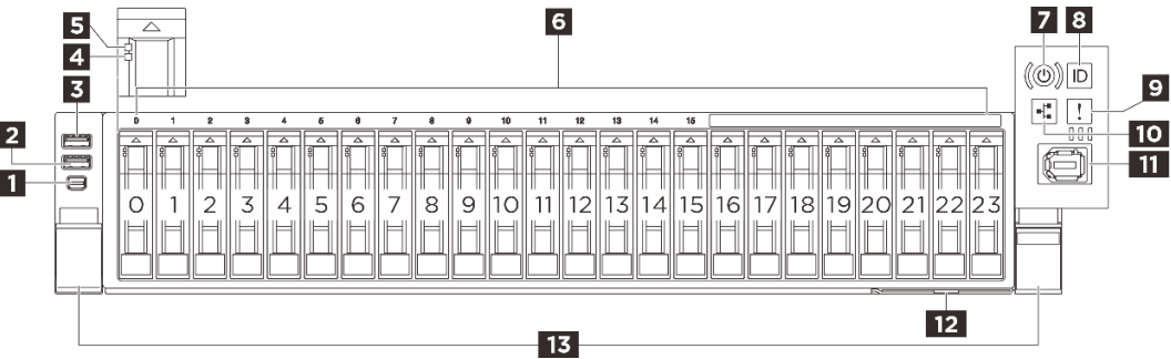
图 2. 配备 2.5 英寸插槽的服务器型号的前视图
