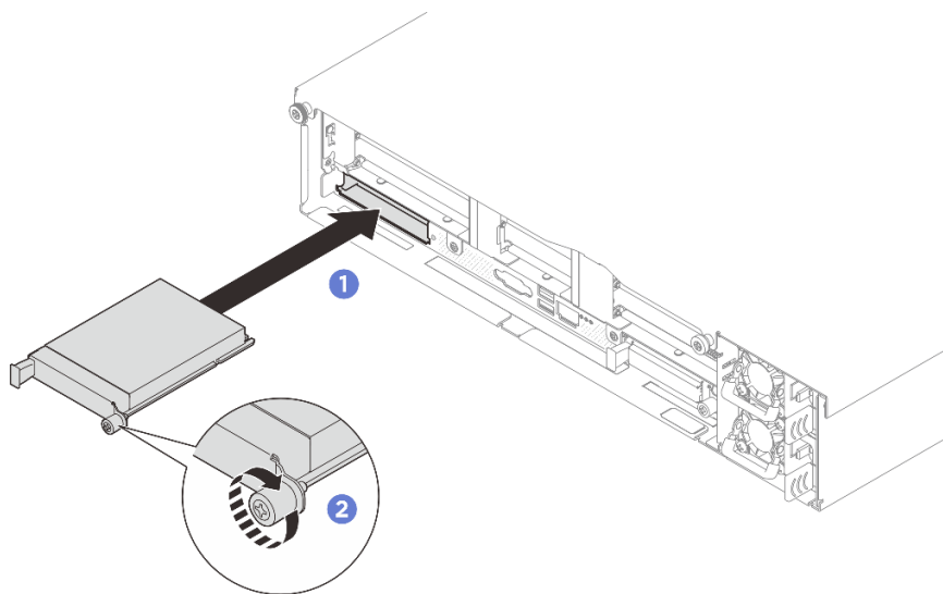
圖例 159. OCP 模組安裝
