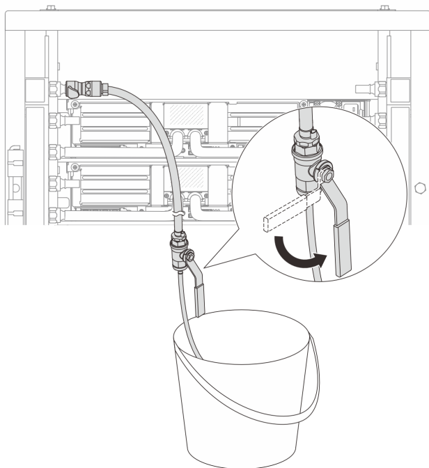
圖例 150. 開啟供應側的洩放閥門
