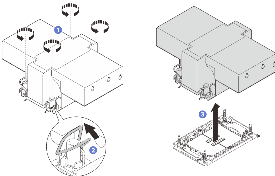
圖例 192. 卸下 2U 效能 PHM
