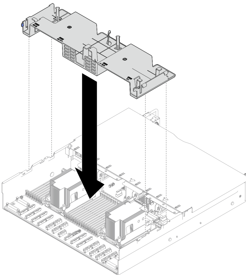
圖例 17. 安裝後方空氣擋板
