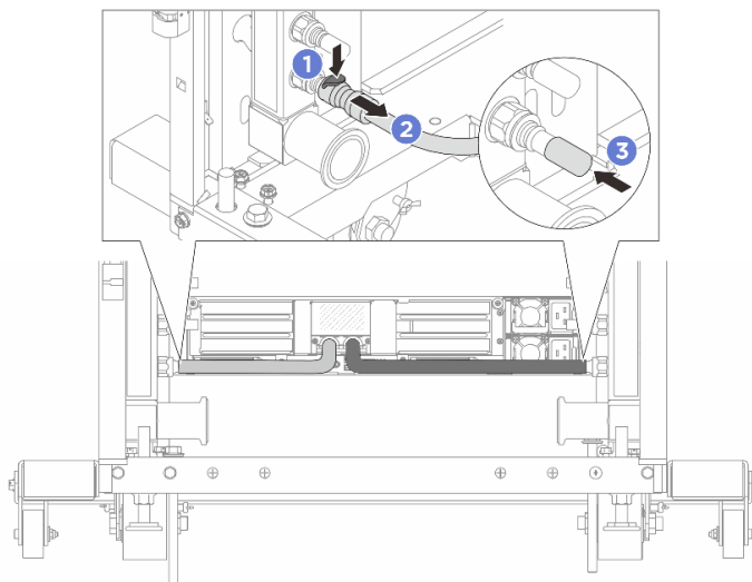
圖例 111. 移除 quick connect 插頭
