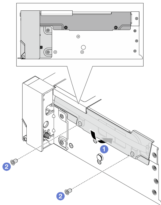
圖例 206. 安裝纜線固定夾
