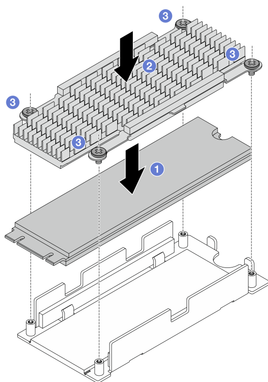
圖例 70. 組裝散熱槽和 M.2 硬碟
