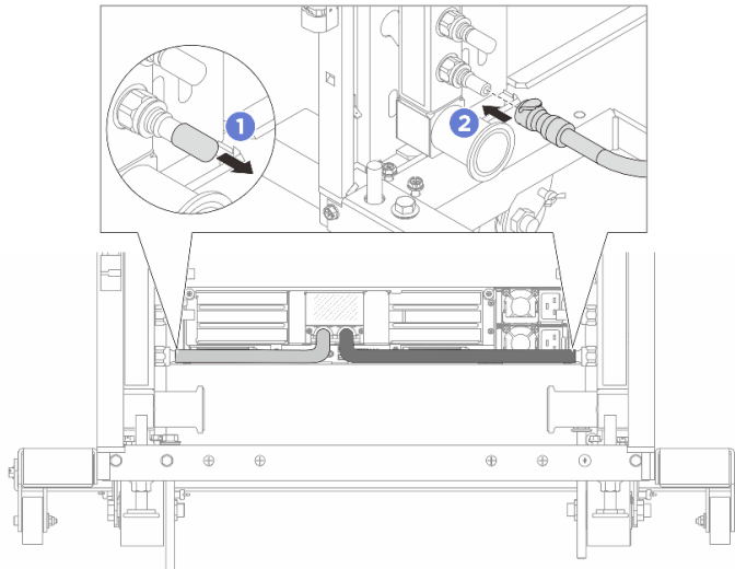
圖例 126. 安裝快速連接插件
