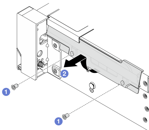
圖例 201. 卸下纜線固定夾
