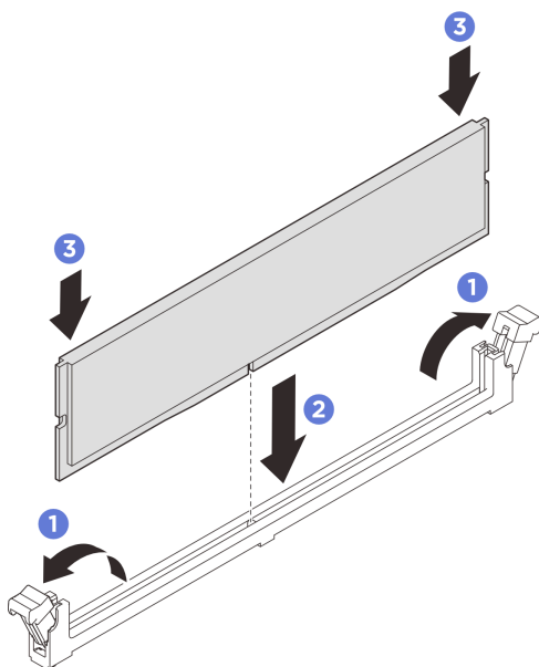
圖例 155. 安裝記憶體模組
