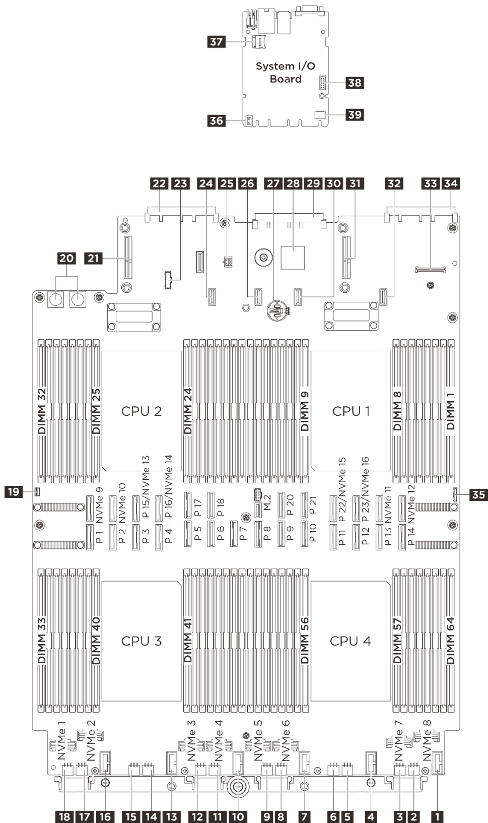
圖例 242. 主機板組件接頭
