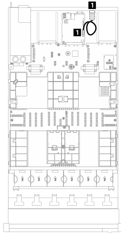
圖例 222. 配備四個 PCIe 擴充卡的伺服器型號的序列埠模組纜線佈線
