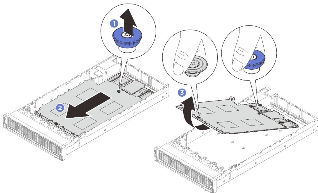
圖例 224. 卸下主機板組件
