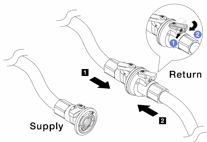
圖例 145. 設施供應至歧管回流
