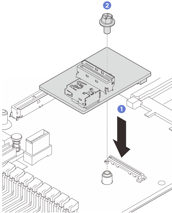
圖例 239. 安裝 USB I/O 板
