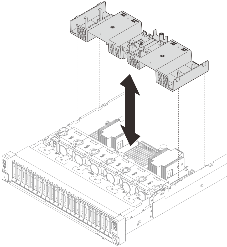
圖例 10. 卸下前方空氣擋板
