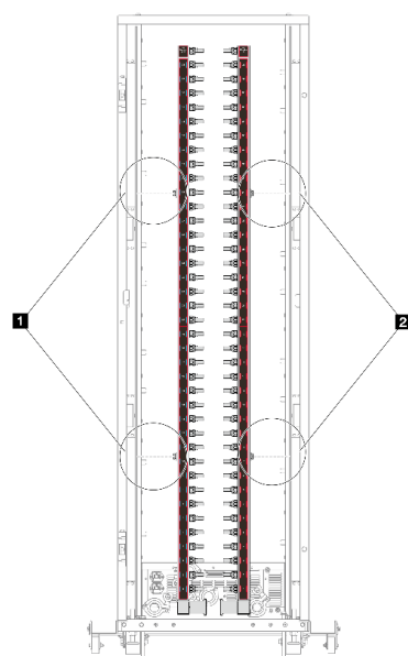
圖例 105. 42U 機架式系統中的歧管
