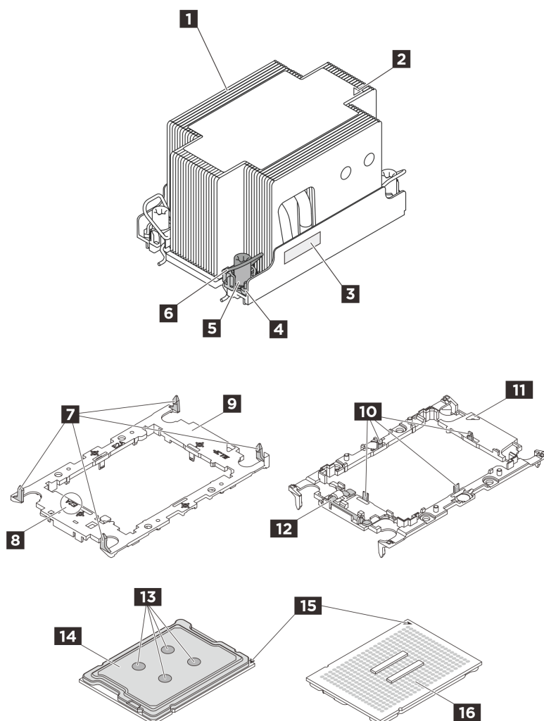
圖例 195. PHM 元件
