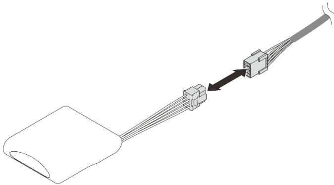
圖例 53. 拔掉快閃記憶體電源模組纜線
