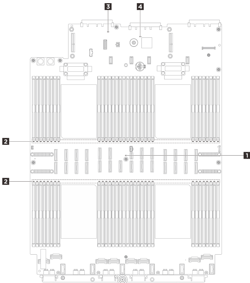
圖例 254. 處理器板 LED
