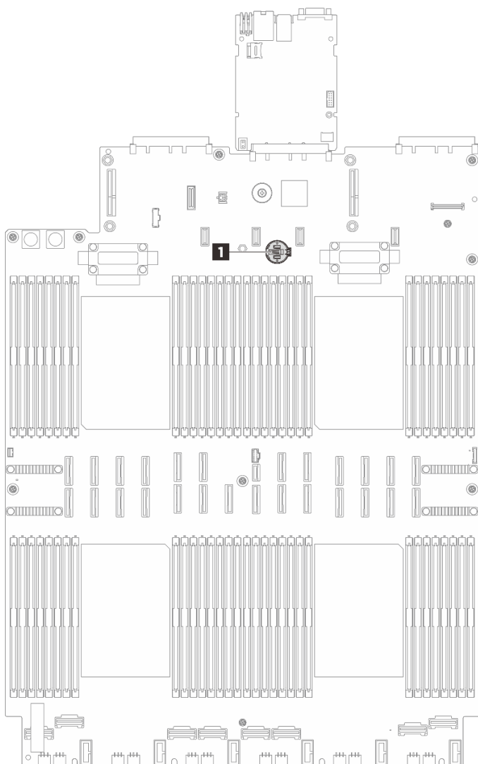
圖例 22. CMOS 電池插槽位置
