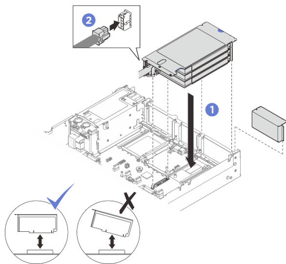
圖例 172. 安裝 PCIe FHHL 擴充卡
