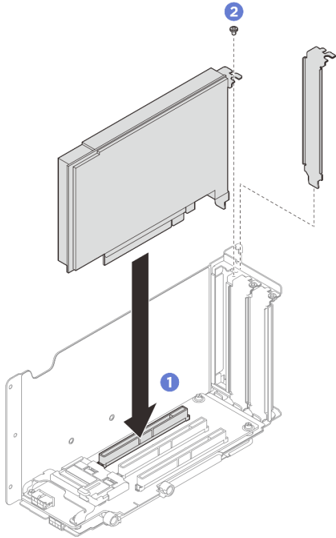
圖例 167. PCIe 配接卡安裝
