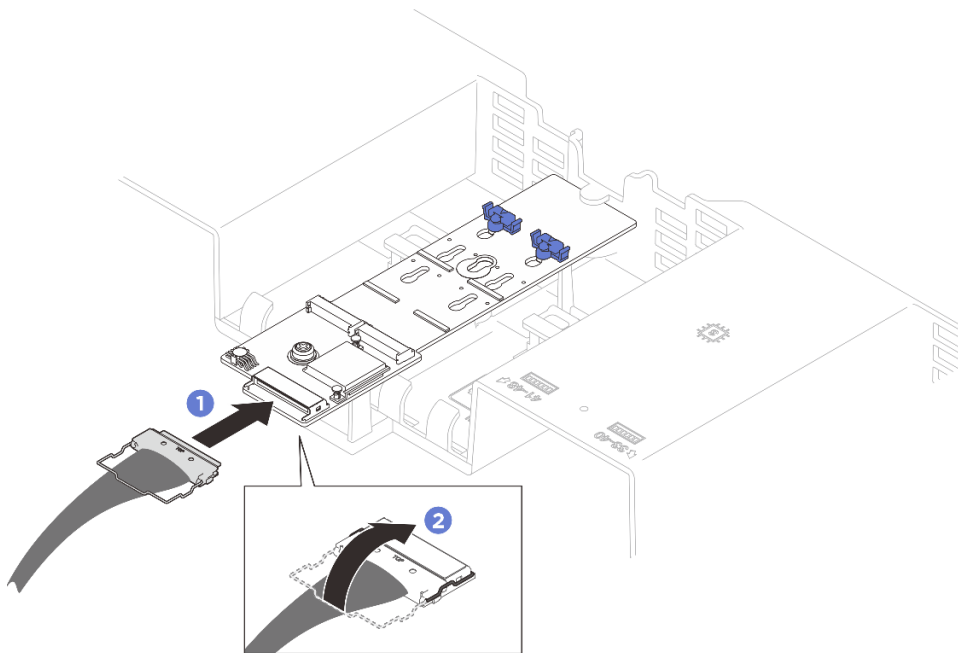
圖例 12. M.2 開機配接卡纜線連接方式
