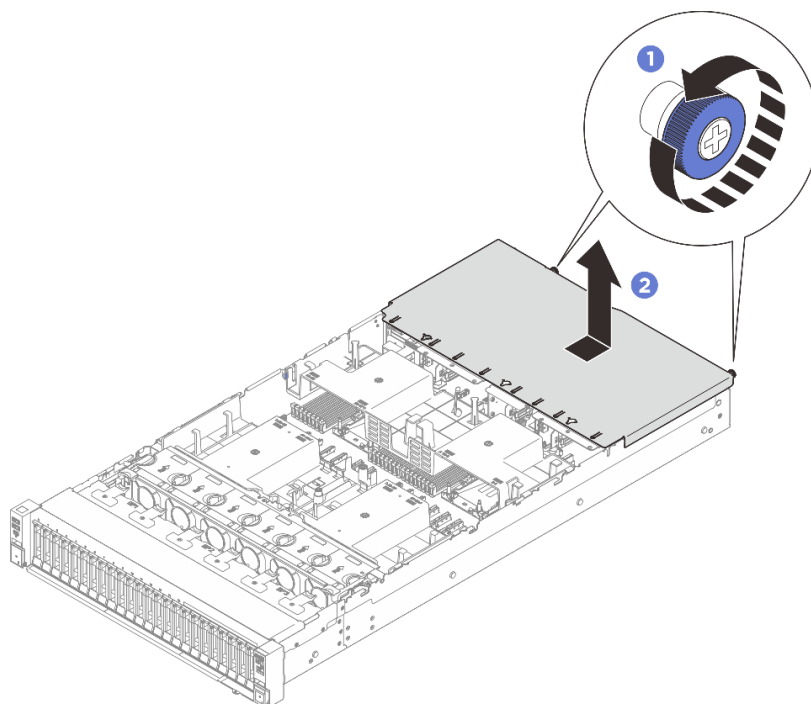
圖例 234. 卸下後方上蓋
