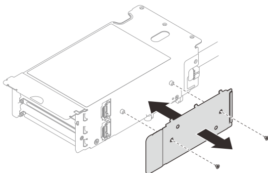
圖例 177. 卸下纜線蓋
