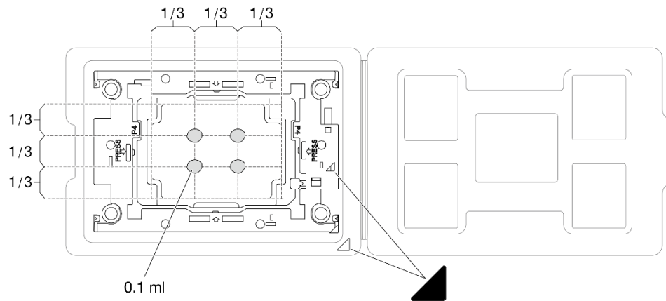
圖例 86. 運送匣中的處理器塗上散熱膏
