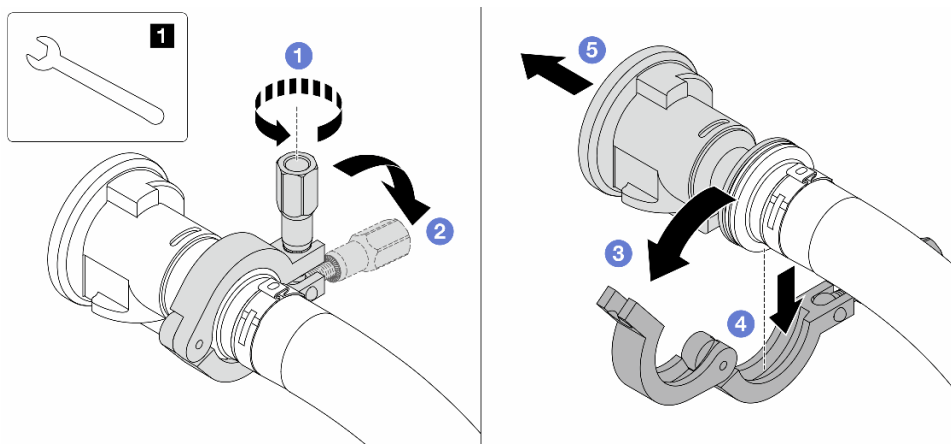
圖例 120. 分開球閥
