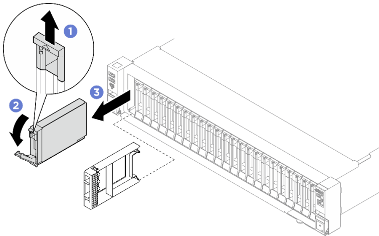
圖例 4. 卸下 2.5 吋熱抽換硬碟
