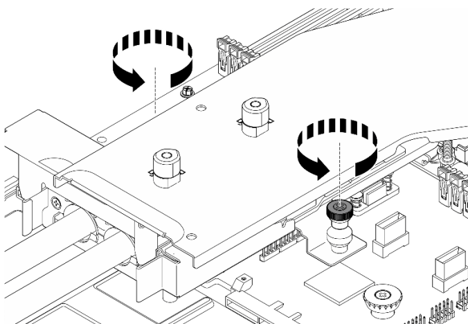
圖例 83. 卸下水冷板組件
