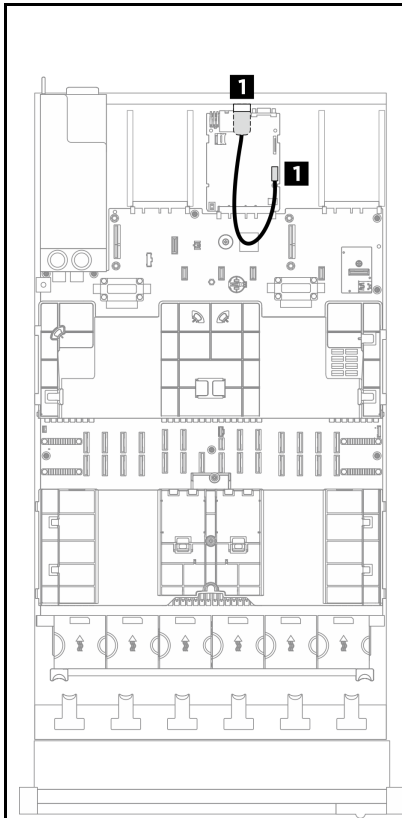
圖例 221. 配備三個 PCIe 擴充卡的伺服器型號的序列埠模組纜線佈線
