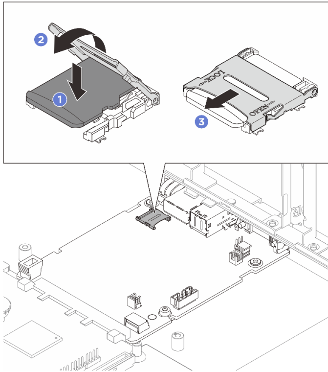
圖例 157. 安裝 MicroSD 卡
