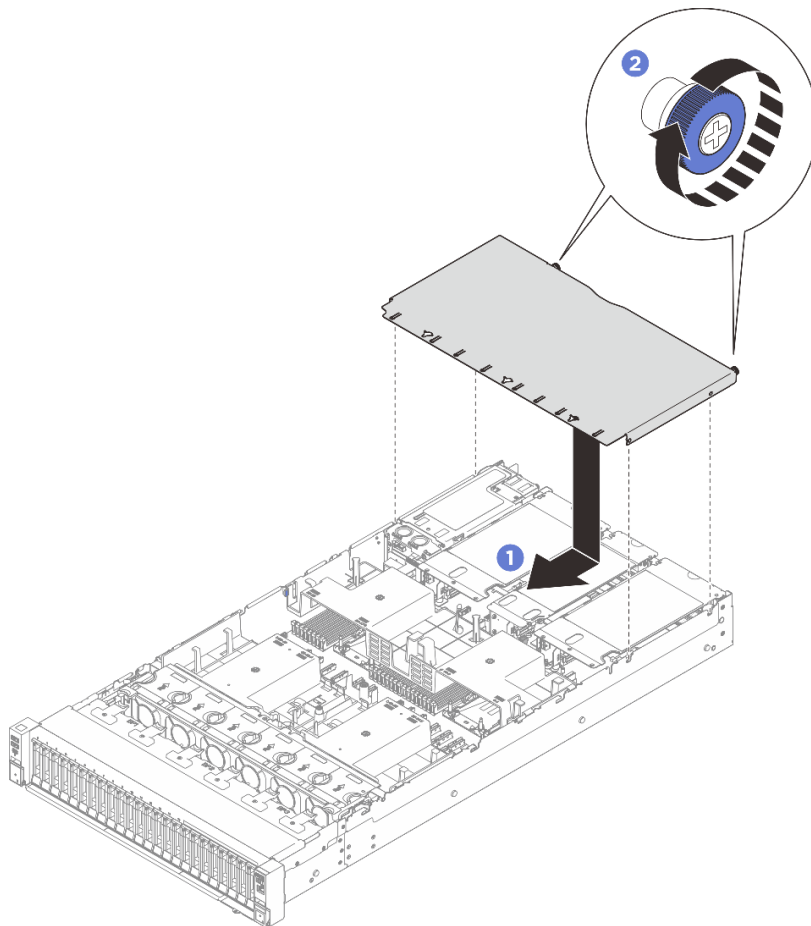
圖例 235. 安裝後方上蓋
