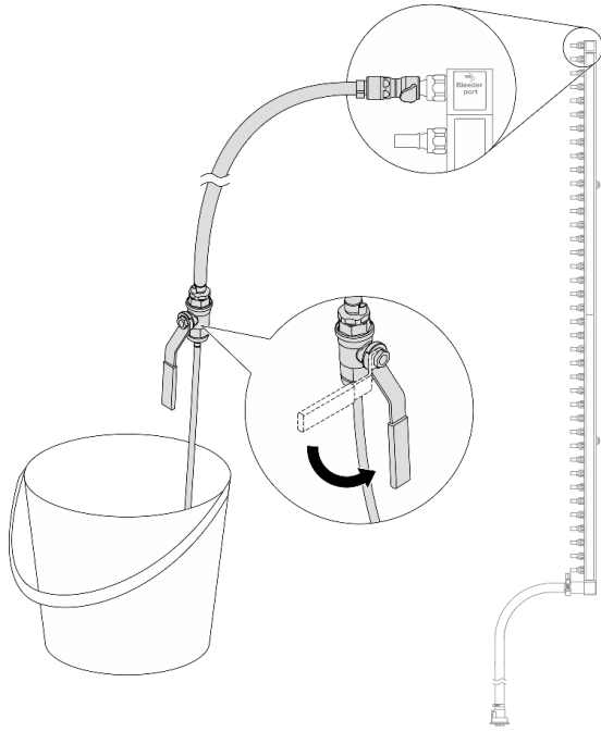
圖例 139. 開啟洩放閥門
