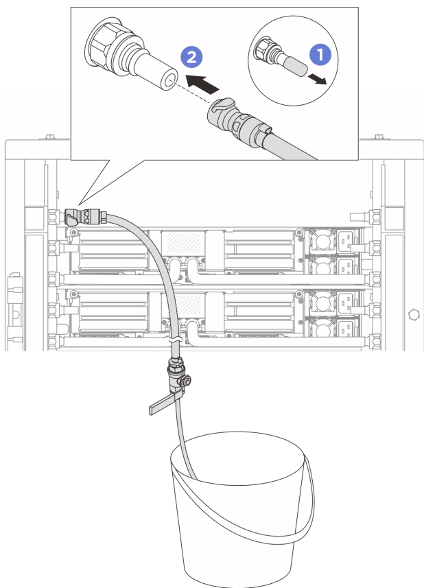
圖例 144. 安裝供應側的洩放套件
