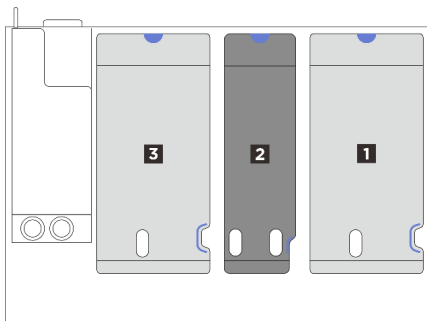
圖例 168. 配備三個 PCIe 擴充卡的伺服器型號
