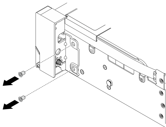
圖例 202. 卸下螺絲
