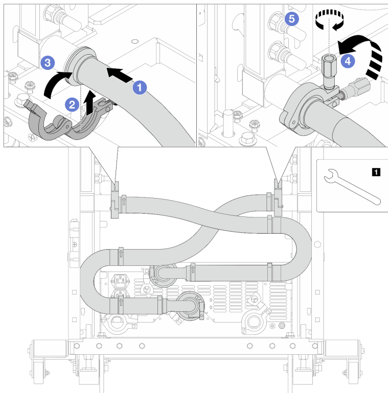
圖例 122. 安裝連接套組
