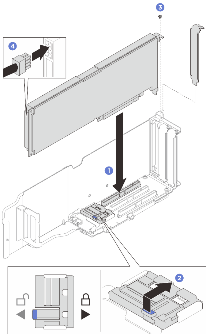
圖例 60. 安裝單寬 GPU 配接卡
