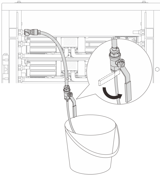
圖例 129. 開啟供應側的洩放閥門
