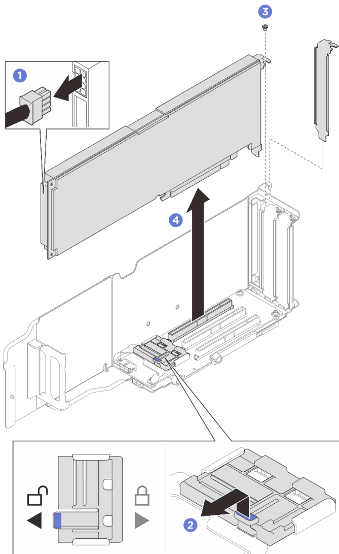
圖例 58. 卸下單寬 GPU 配接卡
