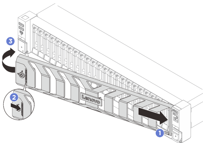
圖例 216. 安裝安全擋板
