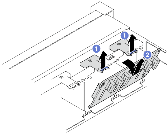
圖例 5. 卸下 2.5 吋硬碟背板
