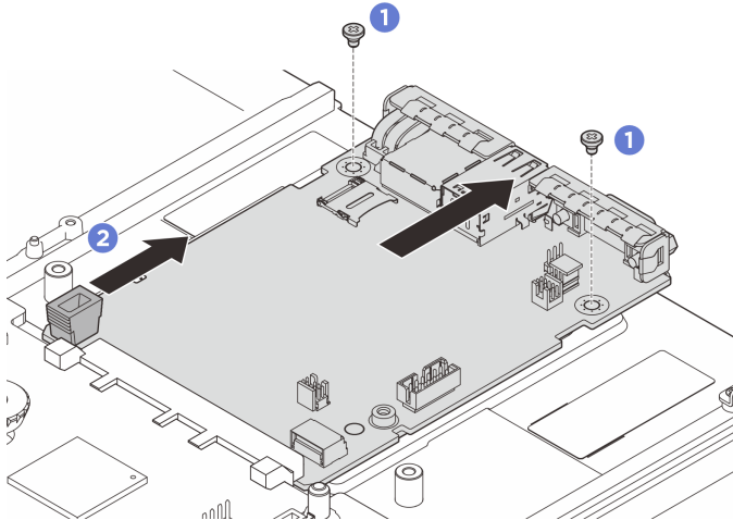
圖例 229. 卸下系統 I/O 板
