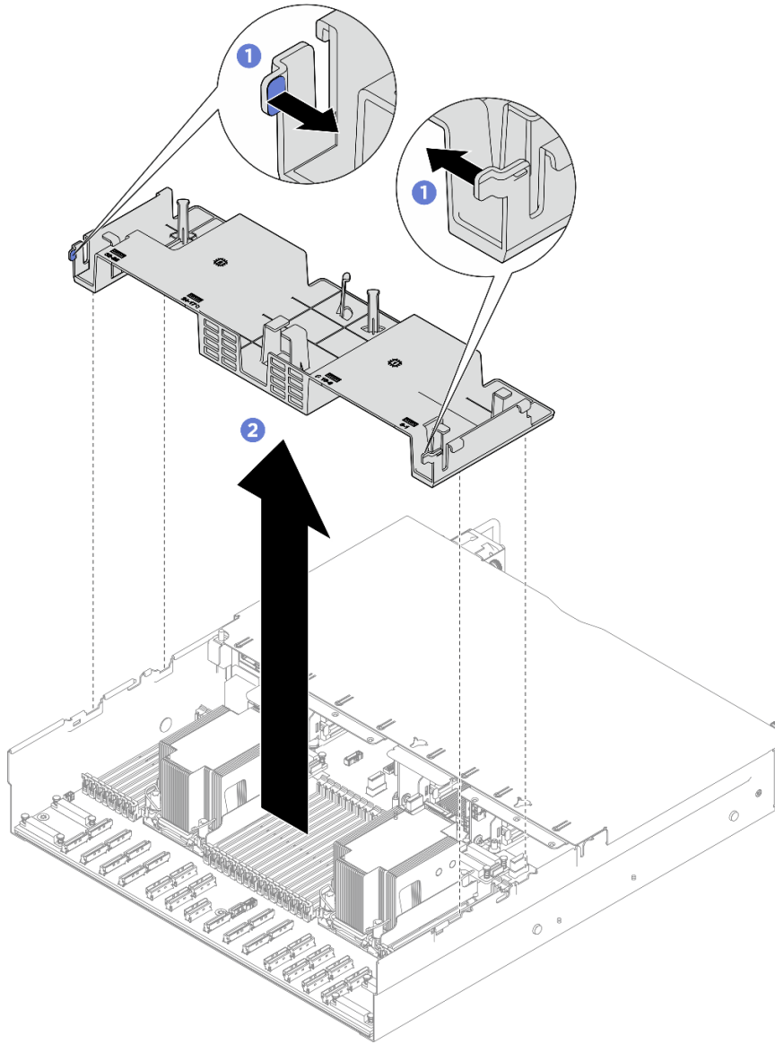
圖例 16. 卸下後方空氣擋板
