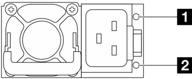
圖例 248. CRPS Premium (CFFv5) 電源供應器上的 LED
