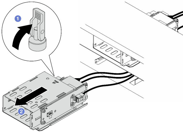
圖例 33. 卸下 E3.S 2T 框架
