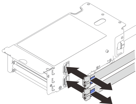
圖例 175. 拔除纜線
