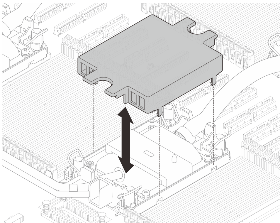
圖例 258. 拆下水冷板蓋
