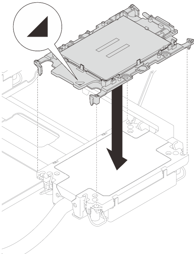
圖例 87. 將處理器安裝到水冷板
