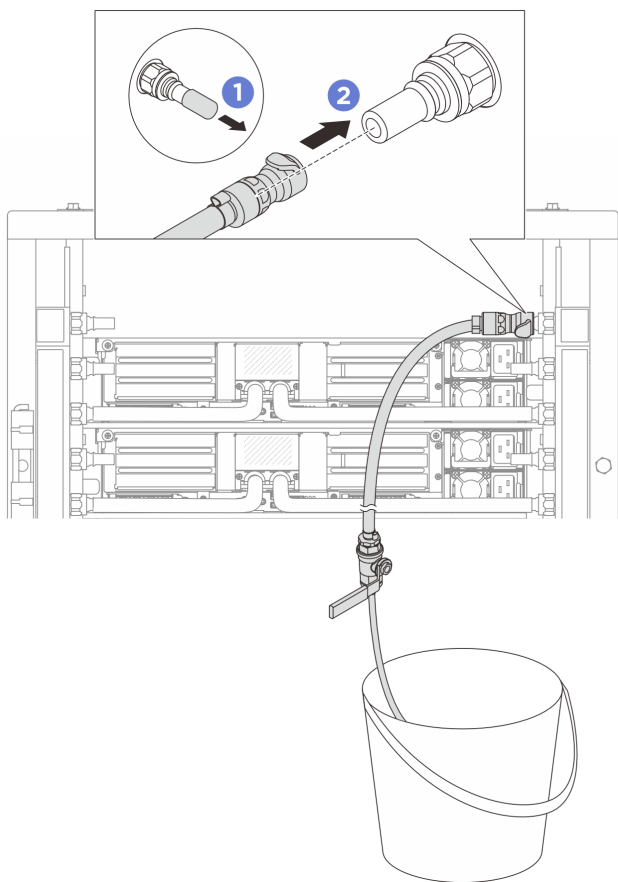
圖例 130. 在回流側安裝洩放套件
