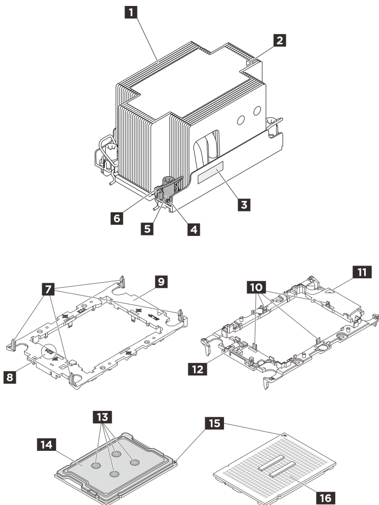
圖例 190. PHM 元件
