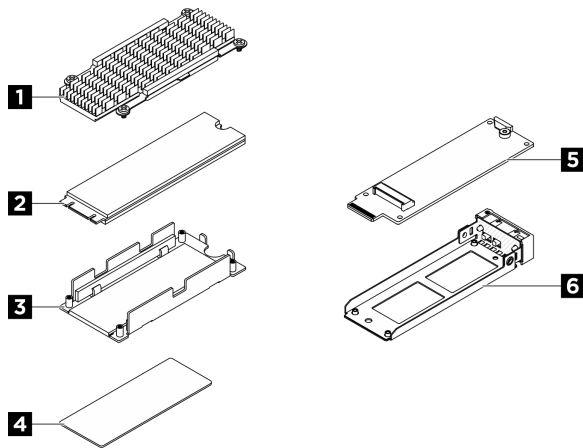
圖例 62. 熱抽換 M.2 硬碟組件的零件
