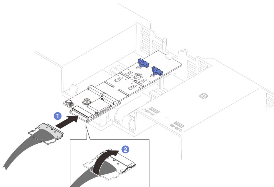
圖例 18. M.2 開機配接卡纜線連接方式
