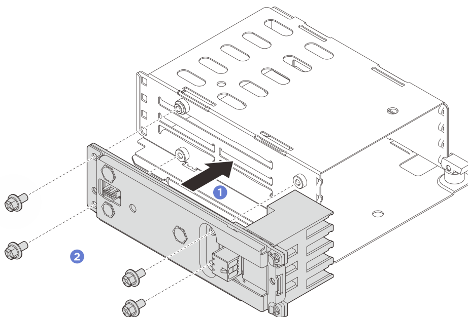
圖例 47. 安裝背板組件
