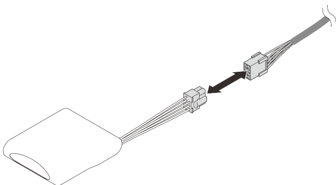
圖例 19. 連接快閃記憶體電源模組纜線
