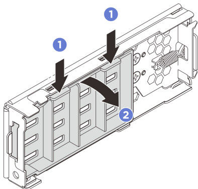
圖例 31. 卸下內板
