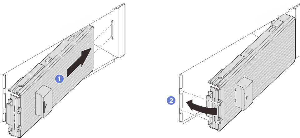
圖例 32. 安裝 E3.S 擋板
