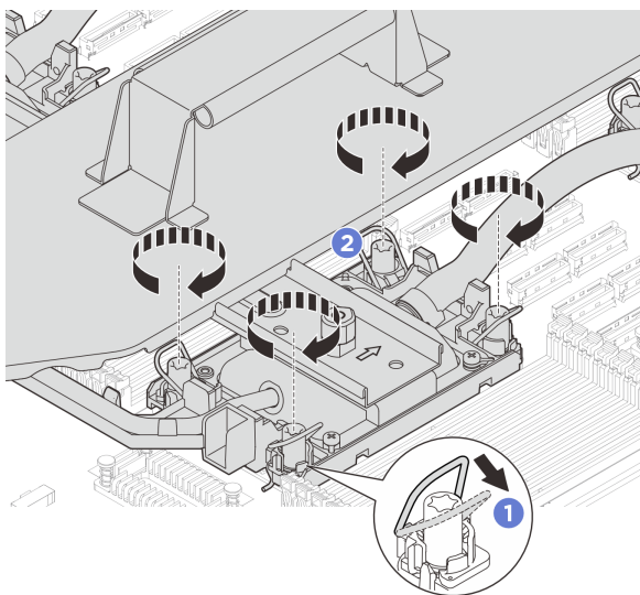
圖例 90. 鎖緊 Torx T30 螺帽
