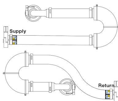
圖例 108. 42U 機架式連接套組
