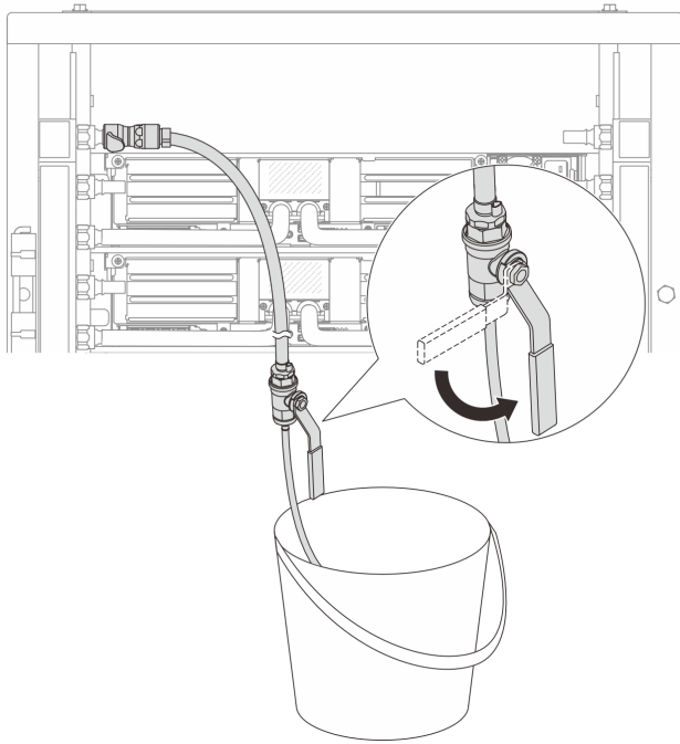
圖例 132. 開啟供應側的洩放閥門
