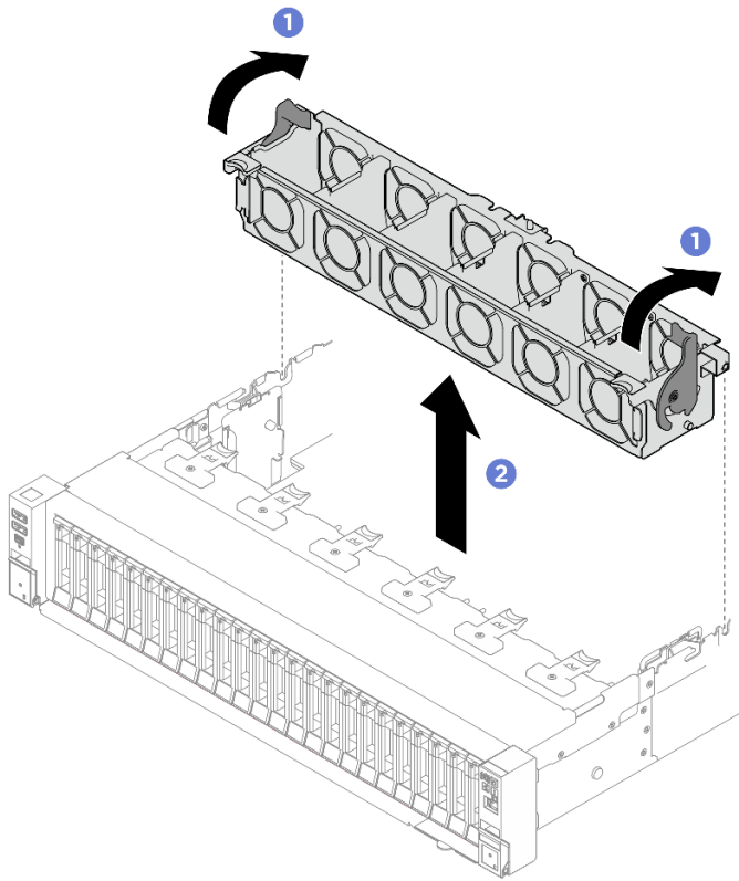
圖例 50. 卸下風扇機盒
