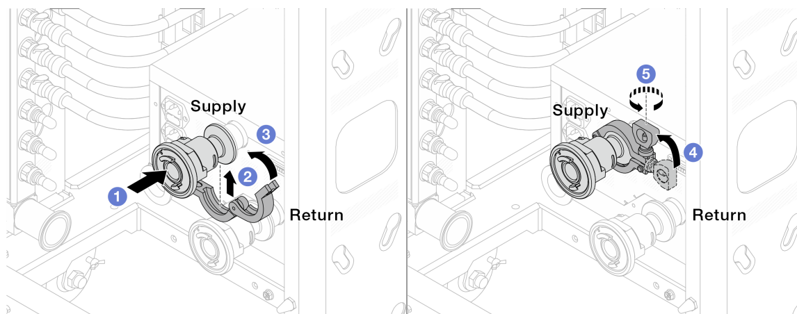
圖例 121. 安裝球閥
