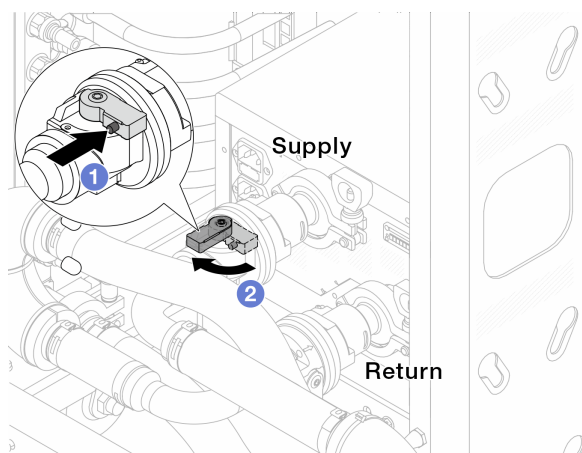
圖例 128. 開啟球閥
