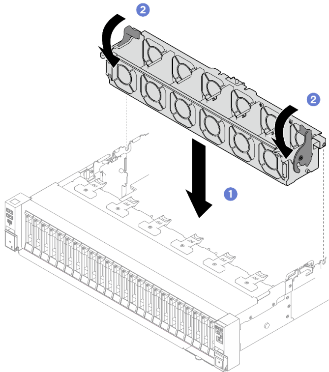
圖例 51. 安裝風扇機盒
