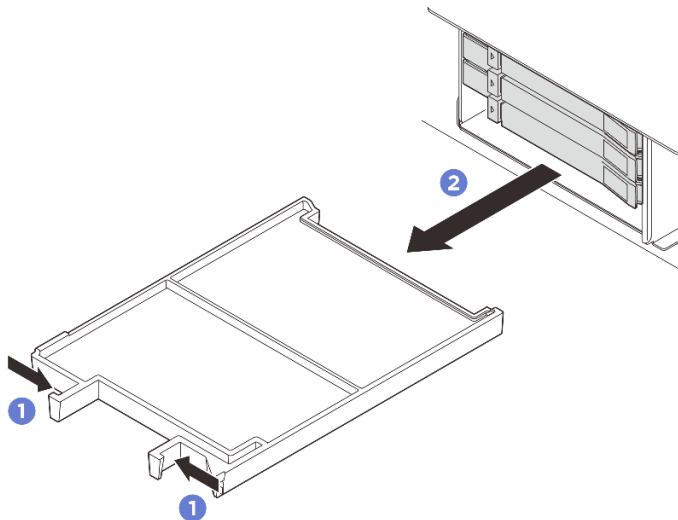
圖例 40. 卸下機槽填充板
