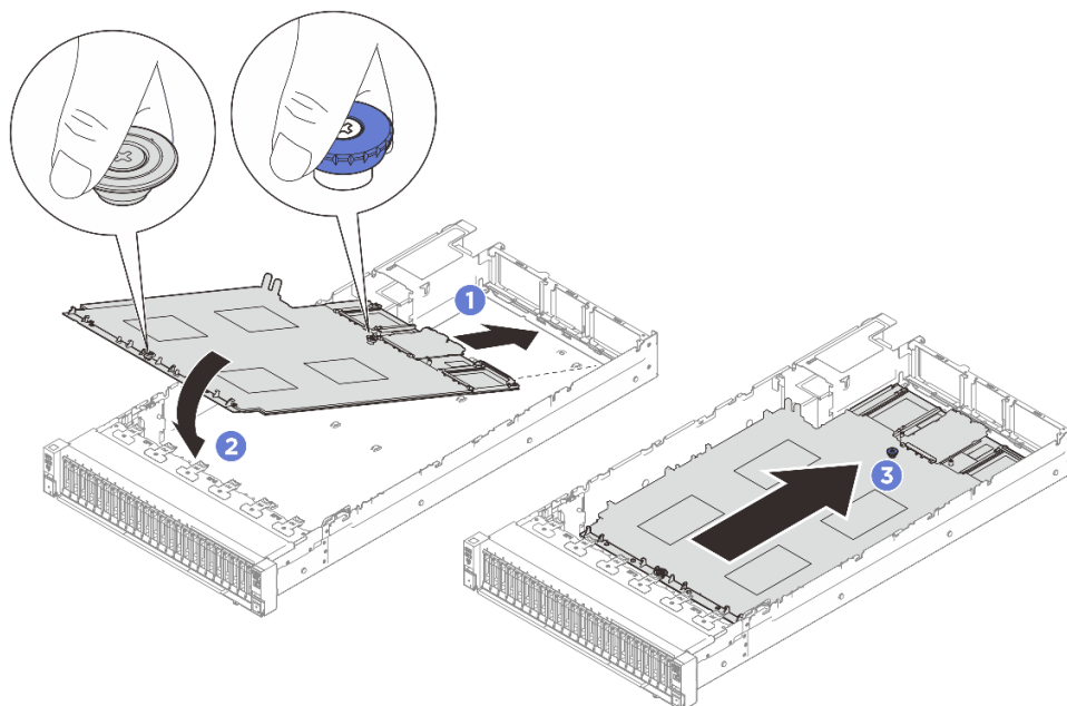
圖例 231. 安裝主機板組件
