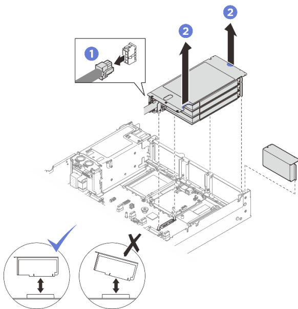
圖例 164. 卸下 PCIe FHFL 擴充卡
