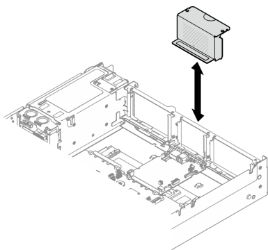
圖例 94. 安裝擴充卡填充板
