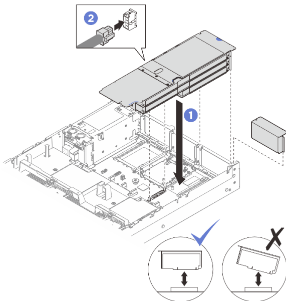
圖例 173. 安裝 PCIe FHFL 擴充卡
