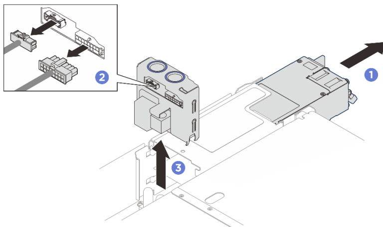
圖例 185. 卸下電源配送板
