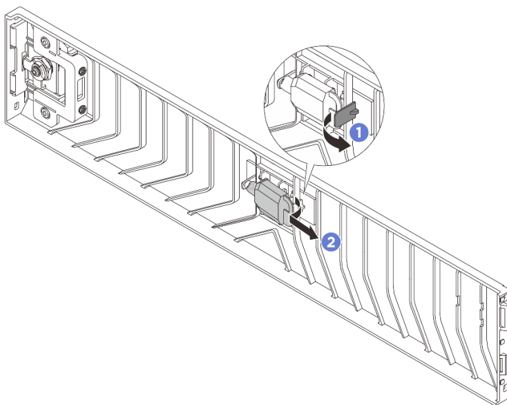
圖例 215. 取出鑰匙
