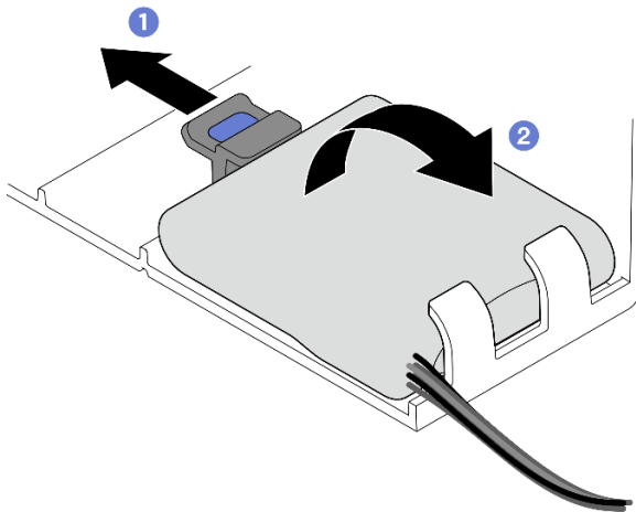
圖例 54. 卸下快閃記憶體電源模組
