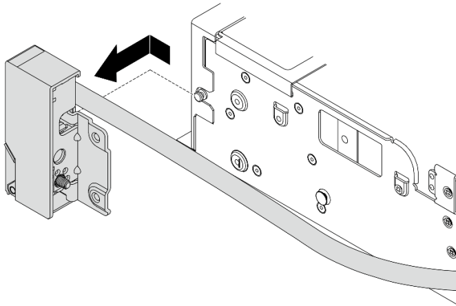
圖例 203. 卸下機架門鎖
