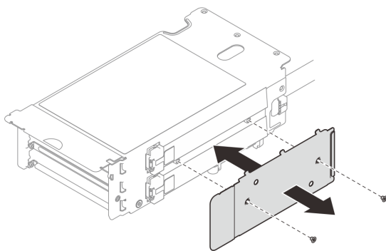
圖例 174. 卸下纜線蓋
