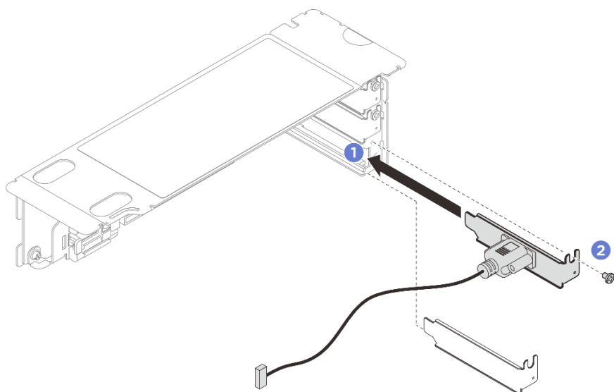
圖例 219. 序列埠模組安裝
