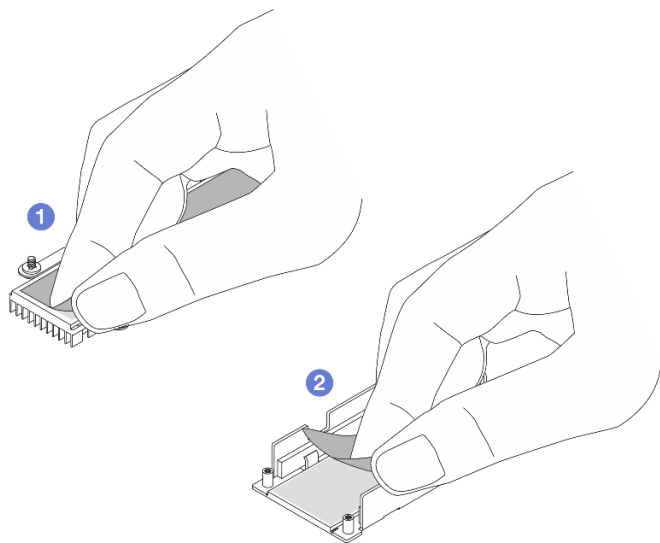
圖例 69. 撕下薄膜
