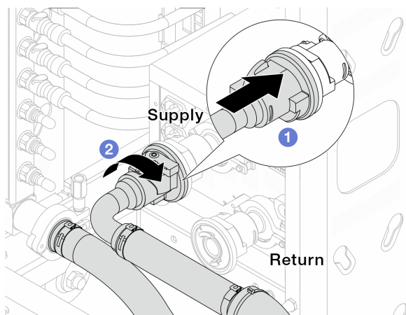
圖例 123. 連接球閥
