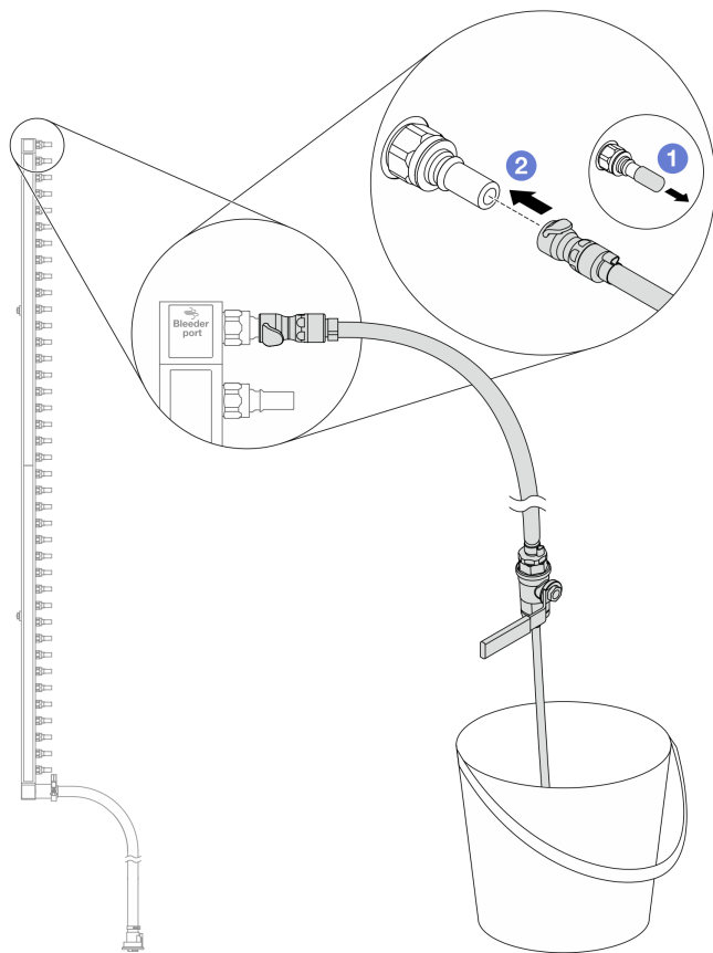
圖例 136. 安裝供應側的洩放套件
