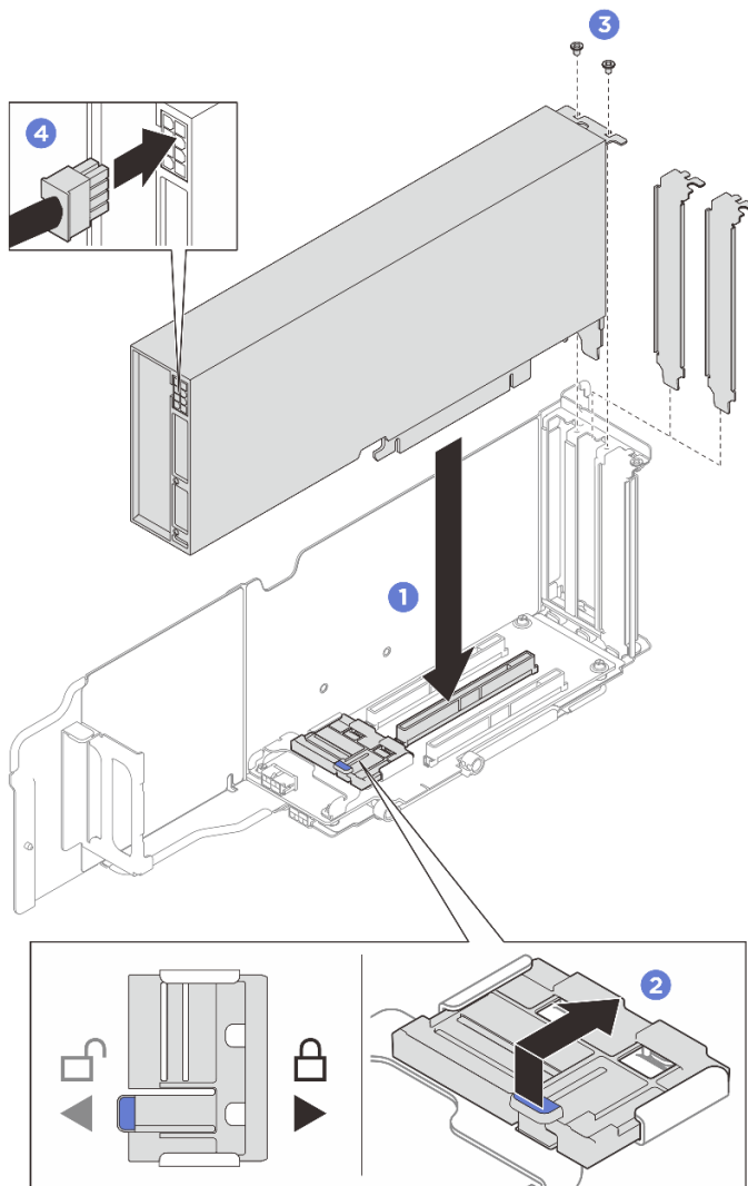
圖例 61. 安裝雙寬 GPU 配接卡
