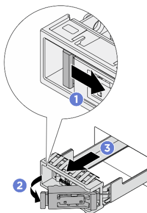
圖例 73. 卸下 M.2 硬碟匣
