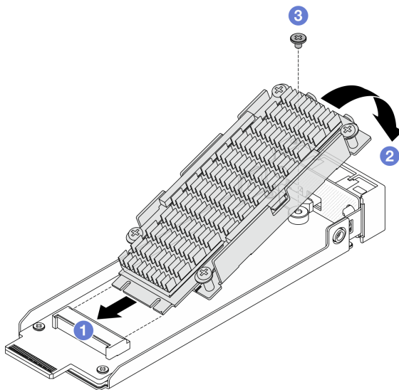
圖例 72. 安裝帶散熱槽的 M.2 硬碟
