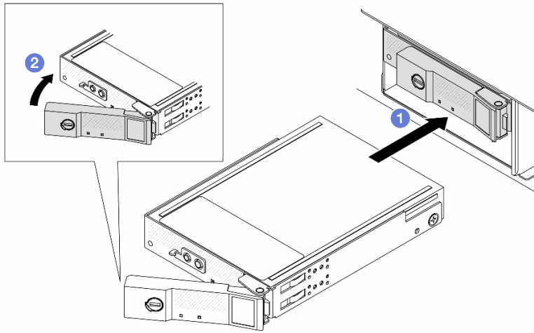
圖例 29. 安裝 E3.S CMM
