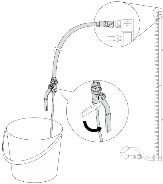
圖例 117. 開啟洩放閥門
