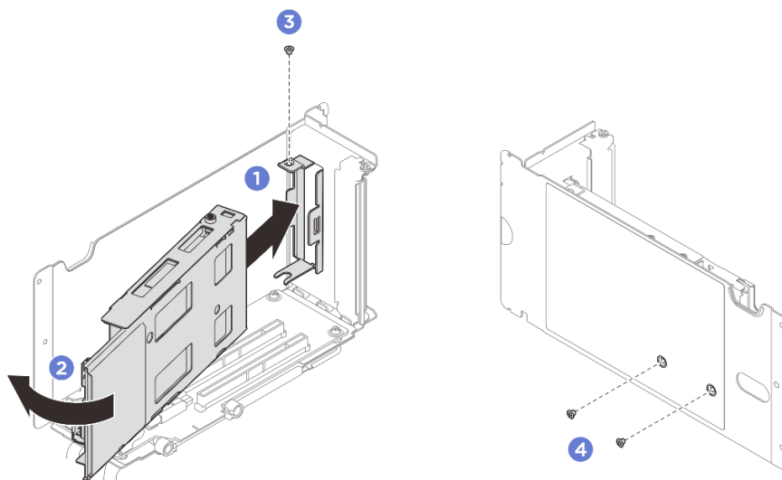
圖例 210. 安裝 M.2 框架
