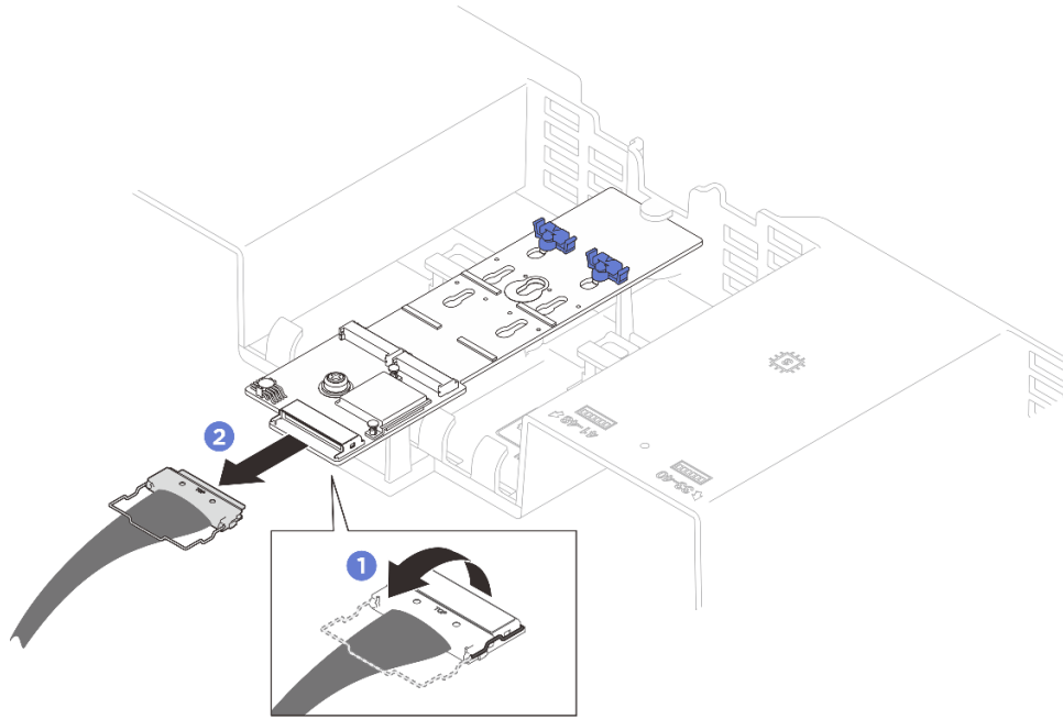
圖例 97. 拔除 M.2 開機配接卡纜線
