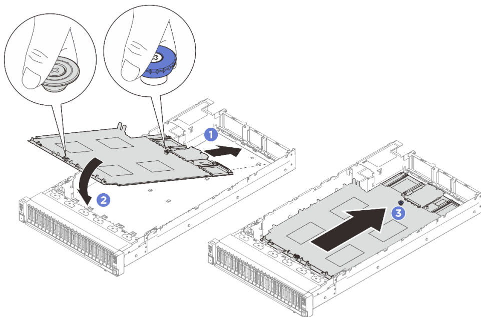
圖例 227. 安裝主機板組件
