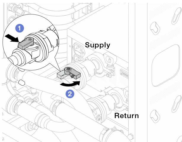
圖例 110. 關閉球閥
