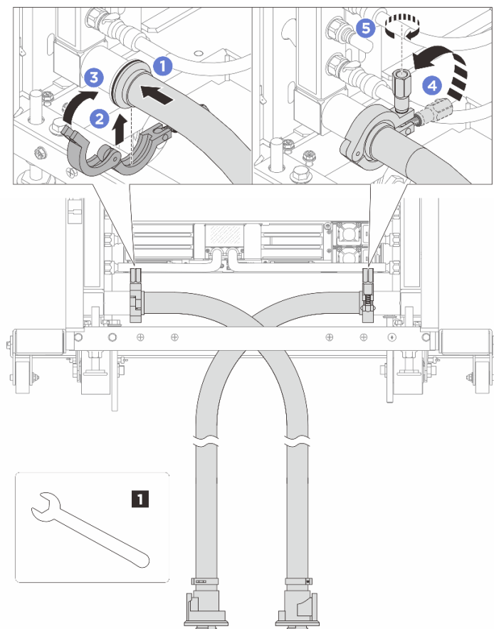
圖例 143. 安裝水管套件
