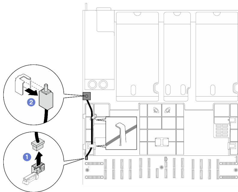
圖例 75. 卸下入侵開關
