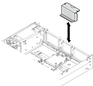
圖例 78. 卸下擴充卡填充板
