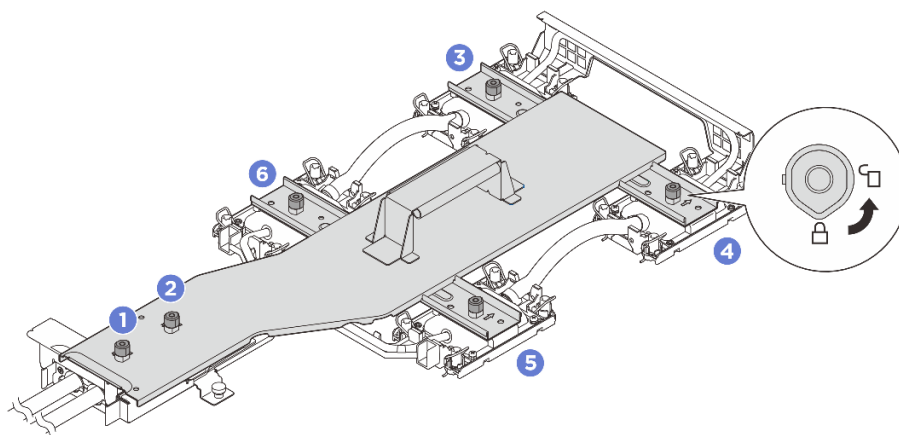
圖例 91. 鬆開水冷板支架
