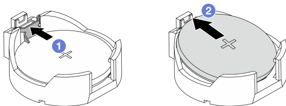
圖例 21. 取出 CMOS 電池
