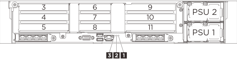
圖例 253. 背面系統 LED
