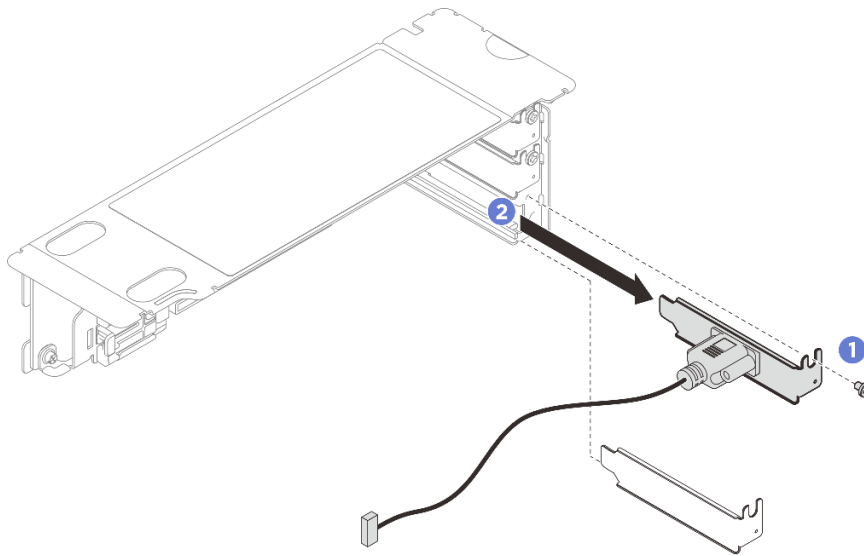
圖例 218. 卸下序列埠模組
