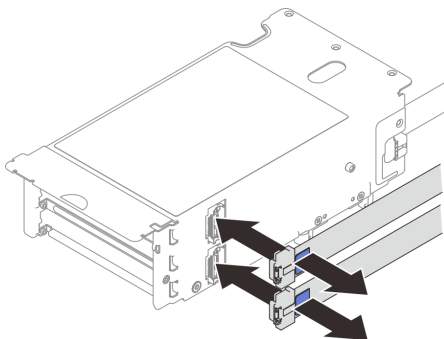
圖例 179. 纜線連接
