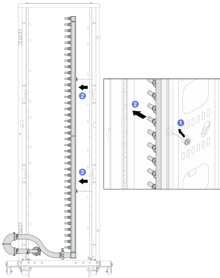
圖例 113. 卸下歧管
