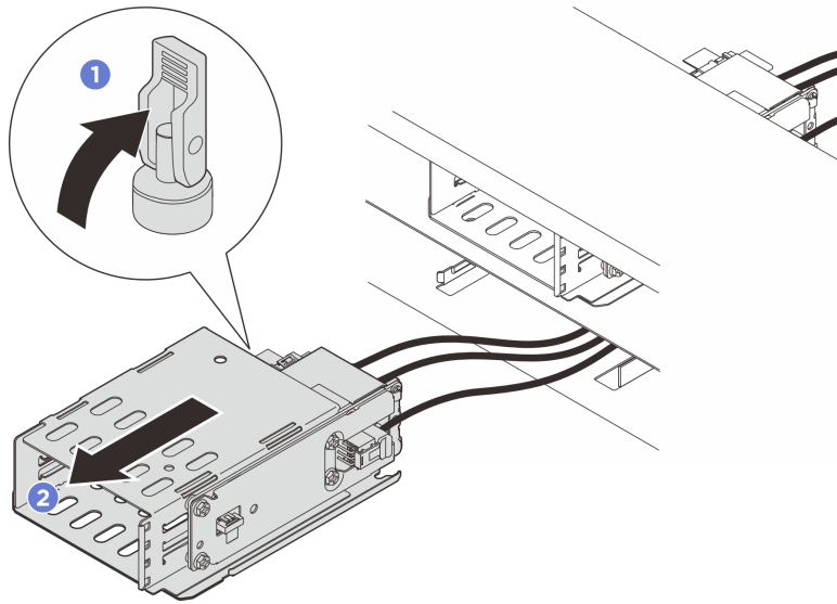
圖例 45. 卸下 E3.S 1T 框架
