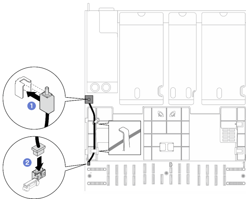
圖例 76. 入侵開關安裝
