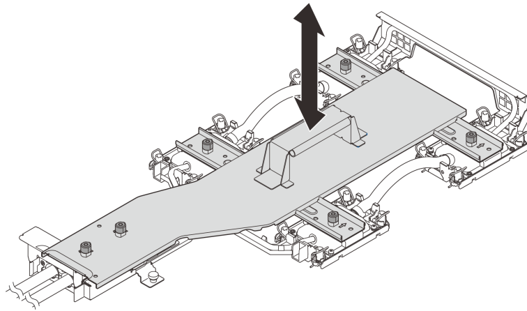
圖例 92. 卸下水冷板支架
