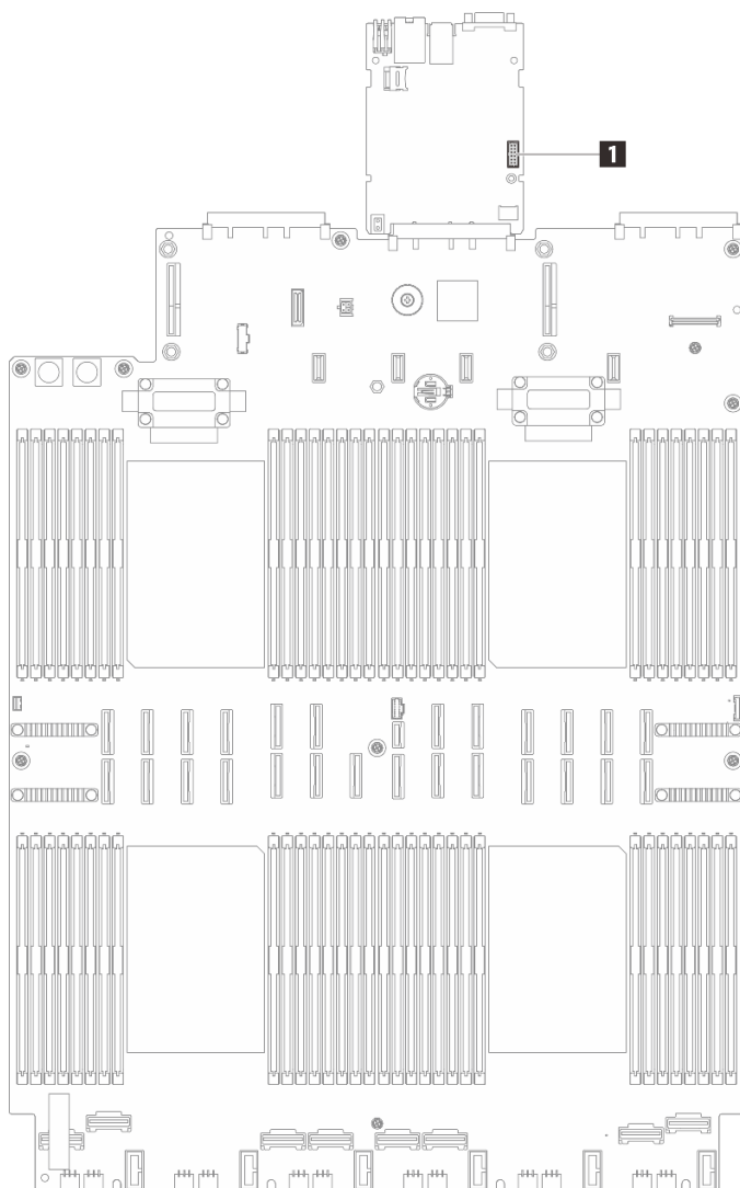
圖例 220. 序列埠接頭位置
