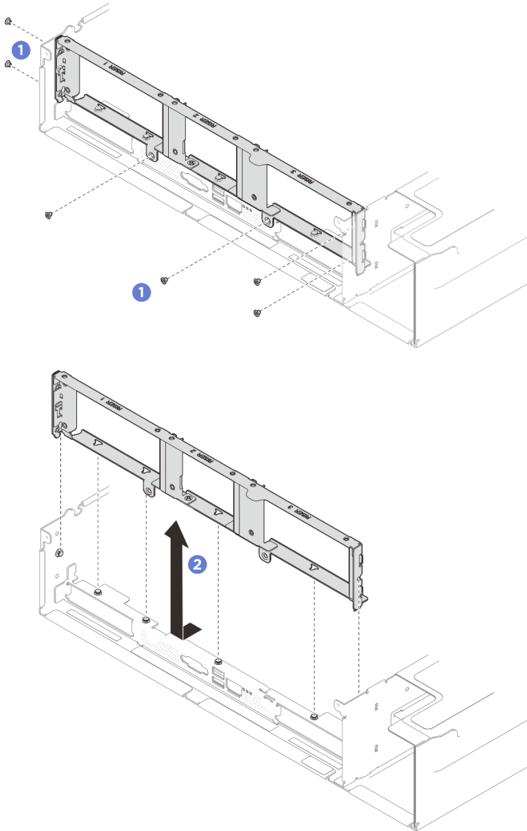
圖例 211. 卸下後壁
