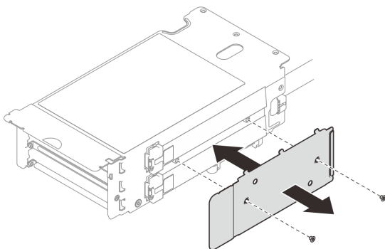
圖例 180. 安裝纜線蓋
