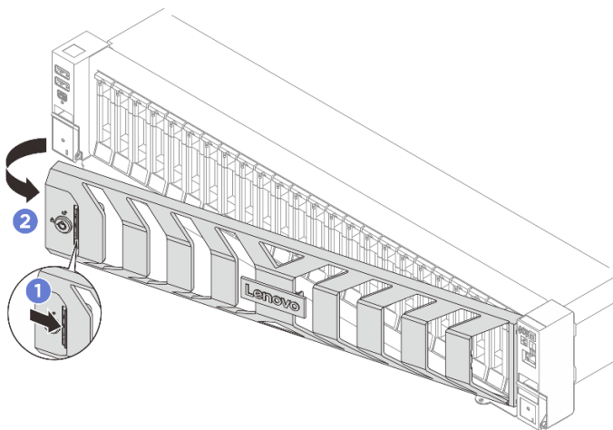
圖例 214. 卸下安全擋板
