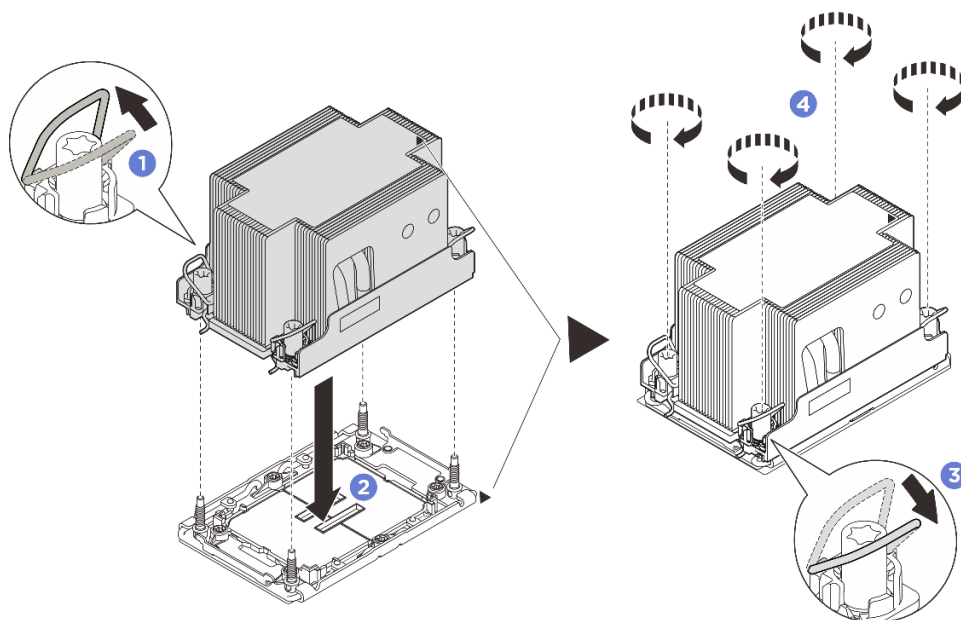
圖例 199. 2U 標準 PHM 安裝
