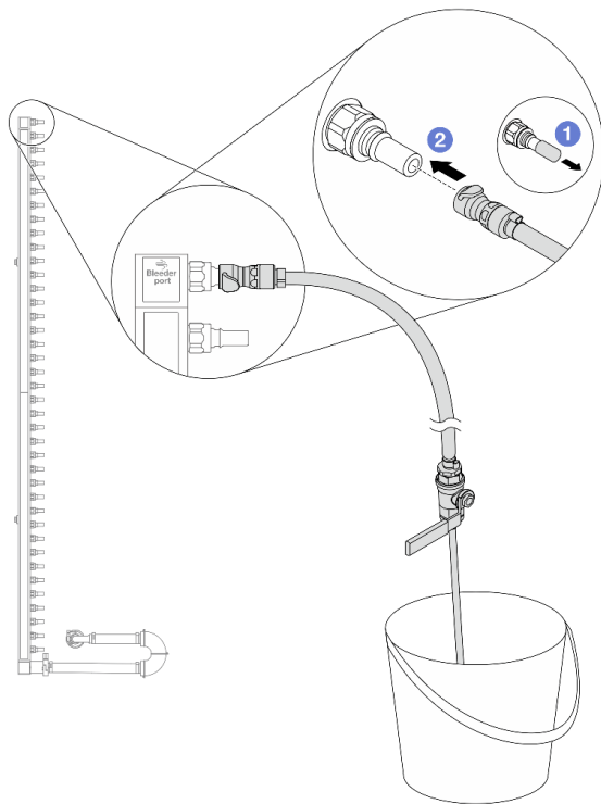
圖例 114. 安裝供應側的洩放套件
