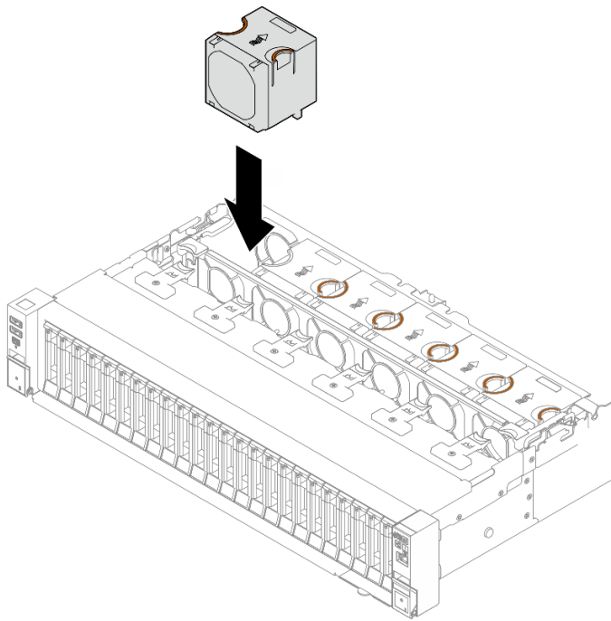
圖例 52. 安裝風扇
