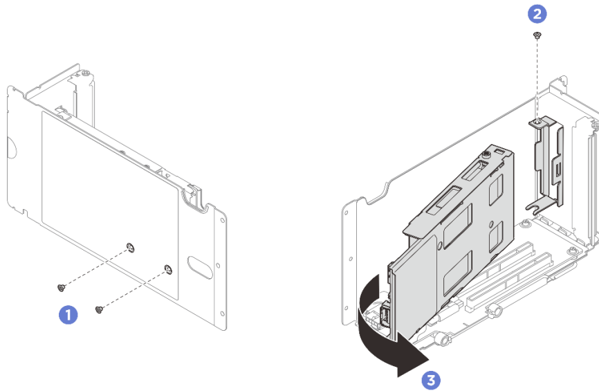
圖例 207. 卸下 M.2 框架
