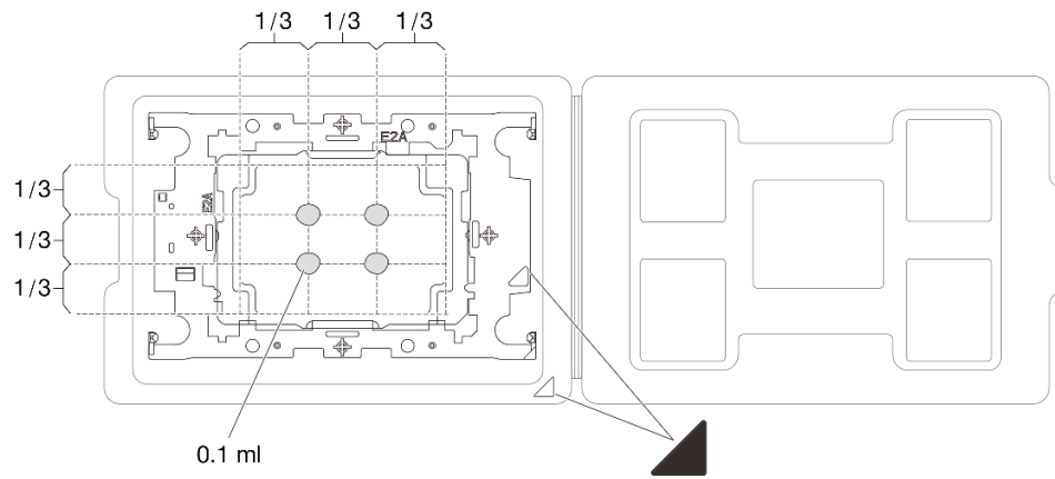
圖例 197. 運送匣中的處理器塗上散熱膏
