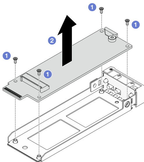
圖例 66. 移除 M.2 轉插卡
