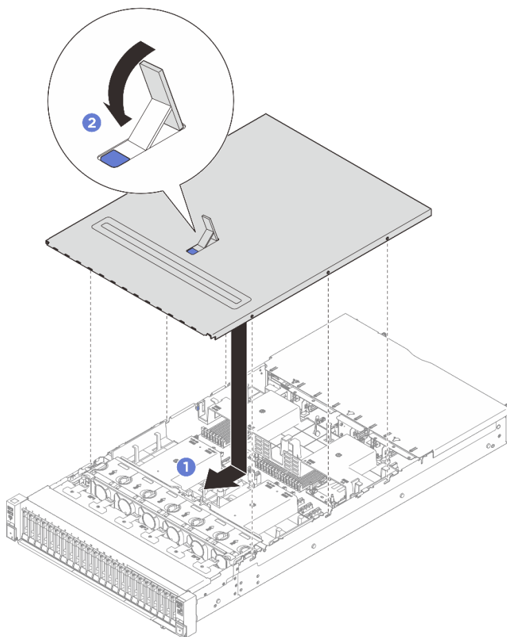
圖例 236. 安裝前方上蓋
