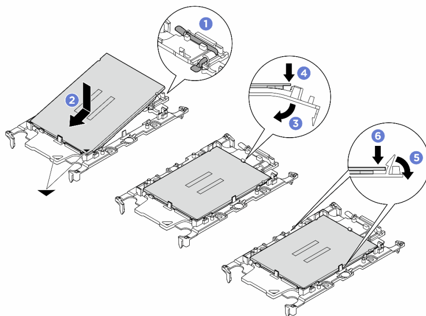
圖例 196. 安裝處理器支架
