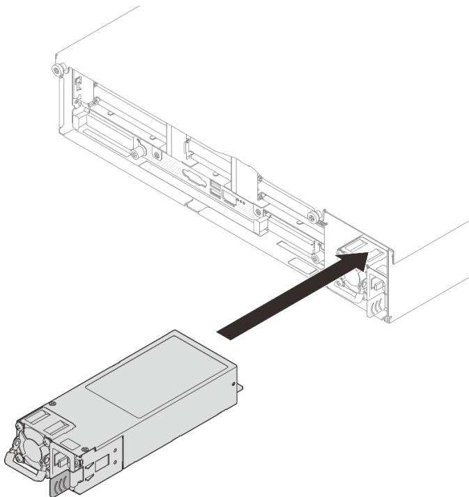
圖例 189. 安裝電源供應器
