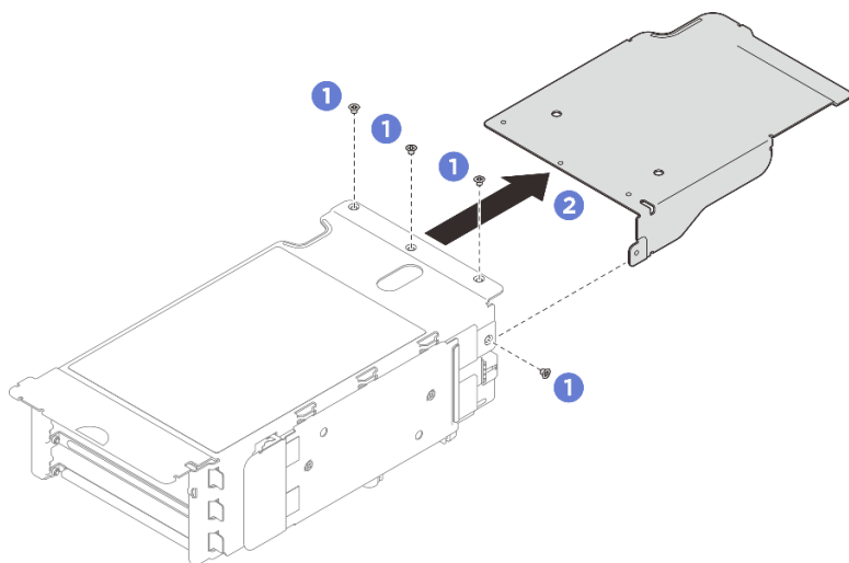
圖例 183. 卸下 PCIe 擴充卡延伸器
