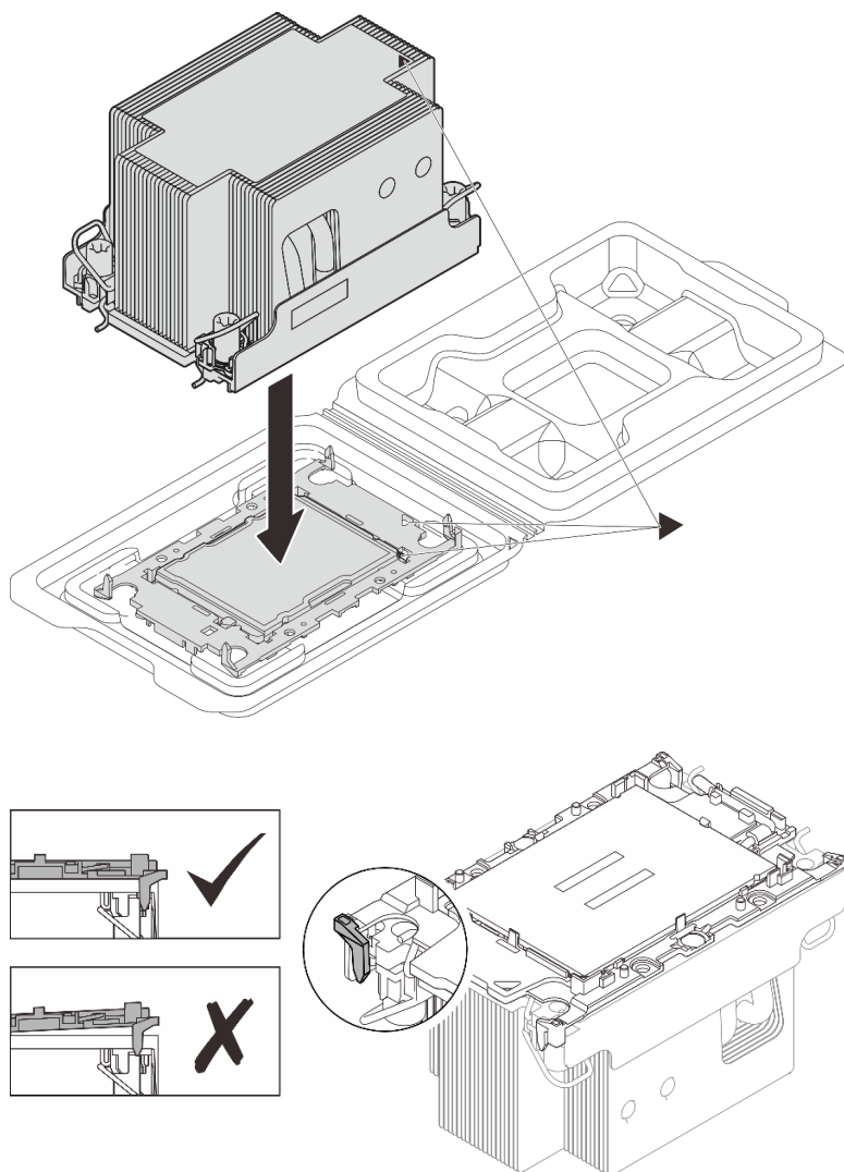
圖例 198. 將 PHM 和處理器裝到運送匣中
