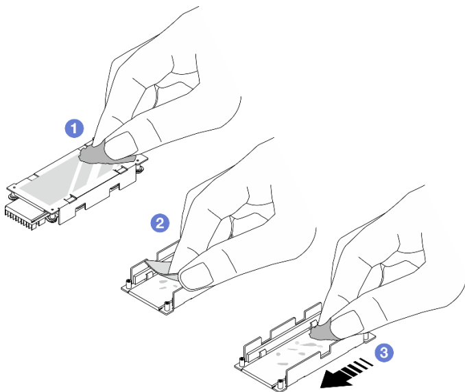
圖例 68. 清潔散熱槽和底板
