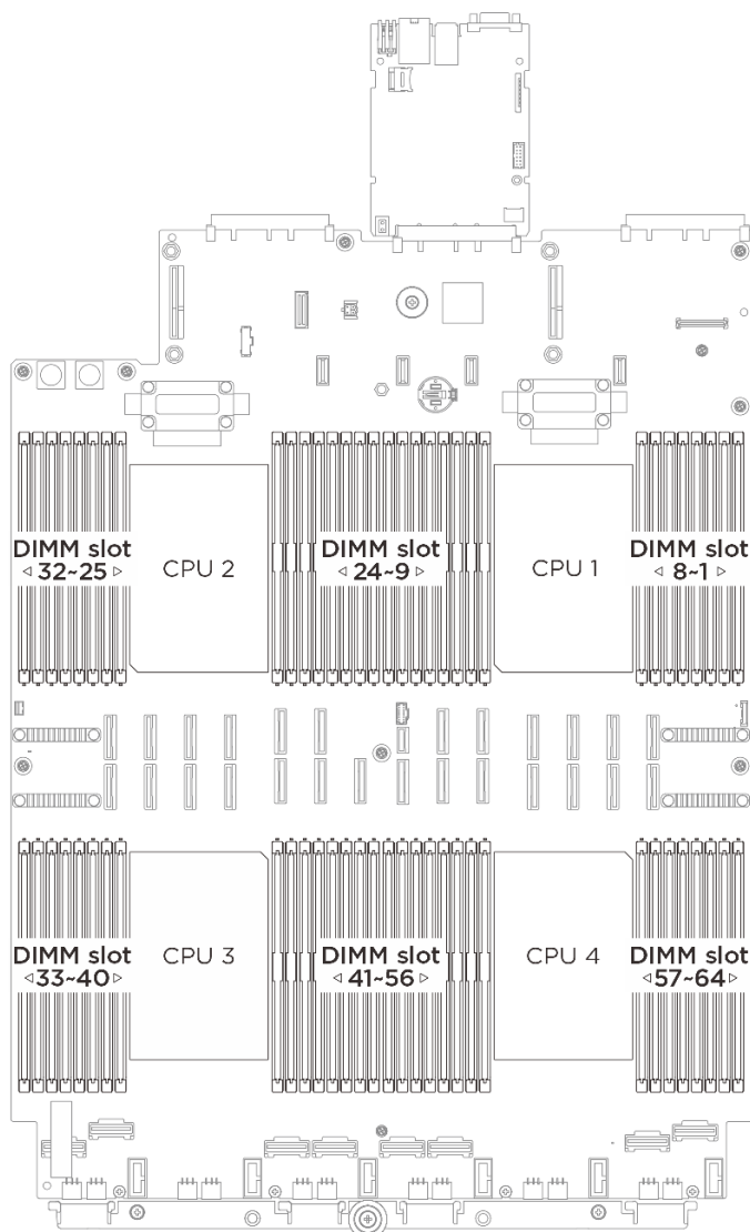
圖例 154. 記憶體模組和處理器佈置
