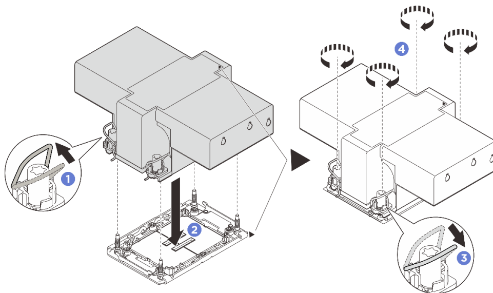
圖例 200. 2U 效能 PHM 安裝
