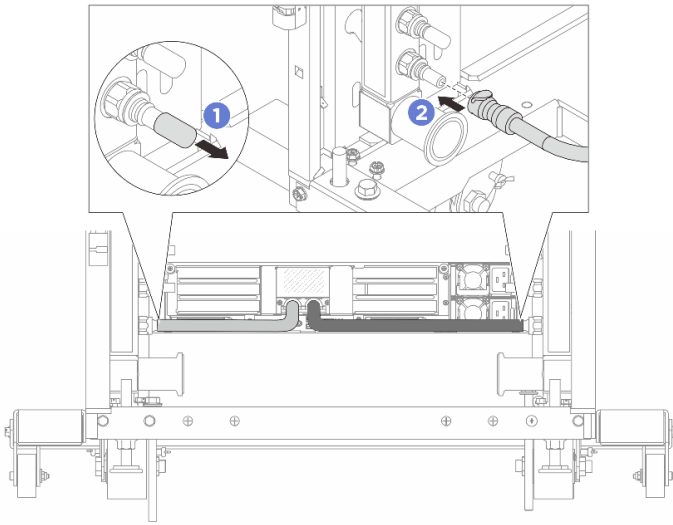
圖例 142. 安裝快速連接插件
