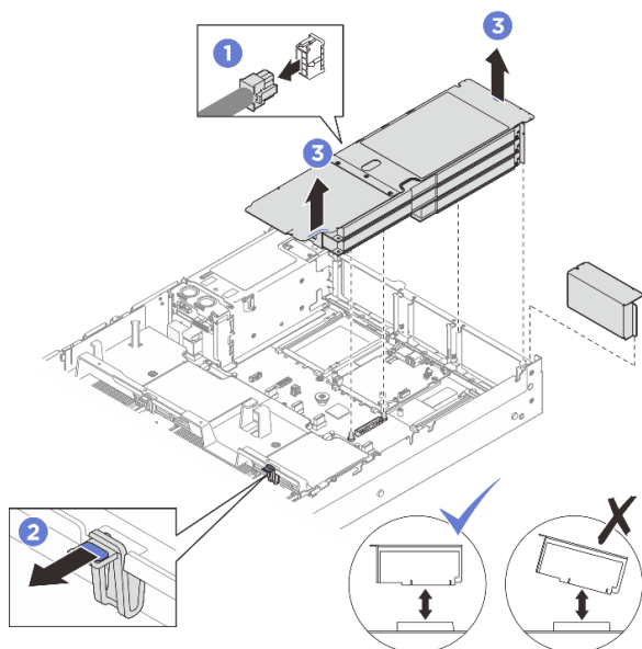
圖例 165. 卸下 PCIe FHFL 擴充卡
