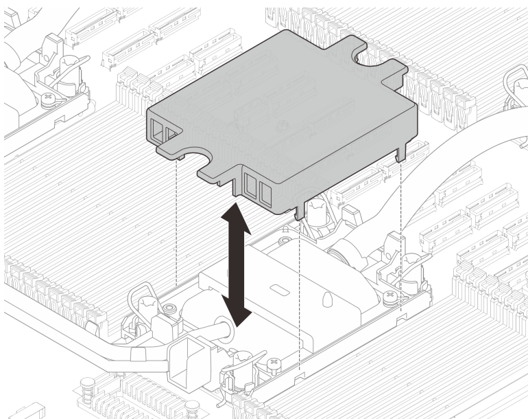
圖例 79. 卸下水冷板蓋
