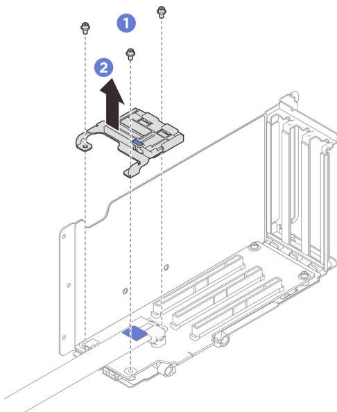
圖例 181. 卸下 PCIe 固定器
