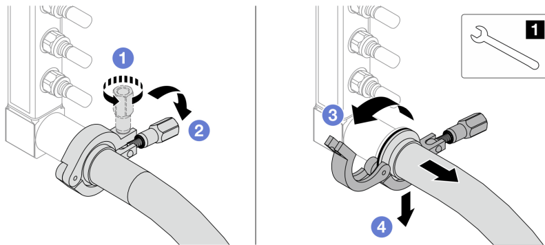
圖例 118. 將歧管與連接套組分開
