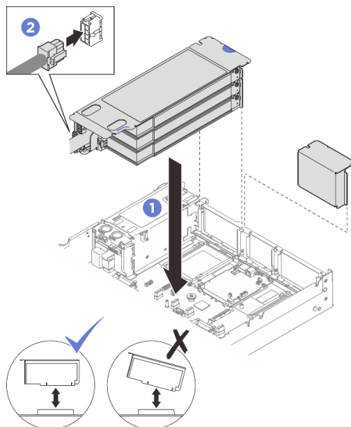
圖例 171. 安裝 PCIe LP 擴充卡 (含電源線)
