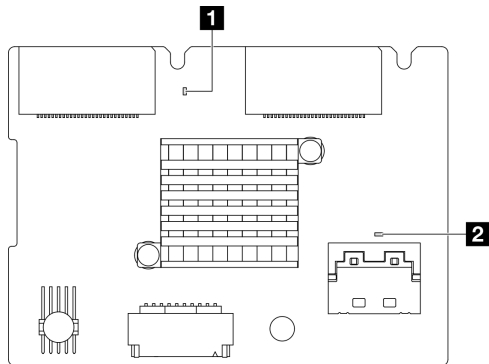
圖例 252. 背面 M.2 開機配接卡 LED
