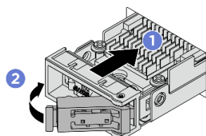
圖例 74. 安裝 M.2 硬碟組件
