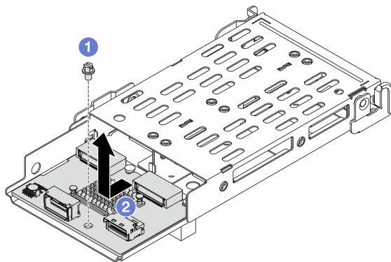
圖例 208. 卸下 M.2 開機配接卡
