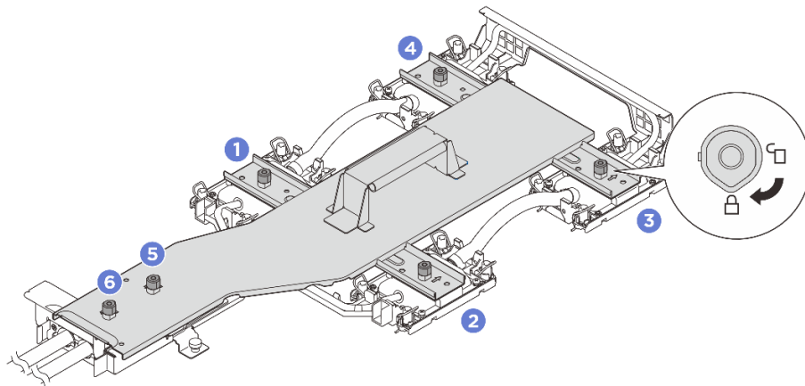
圖例 81. 固定水冷板支架
