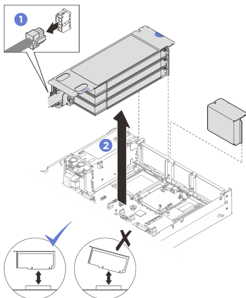
圖例 163. 卸下 PCIe LP 擴充卡 (含電源線)
