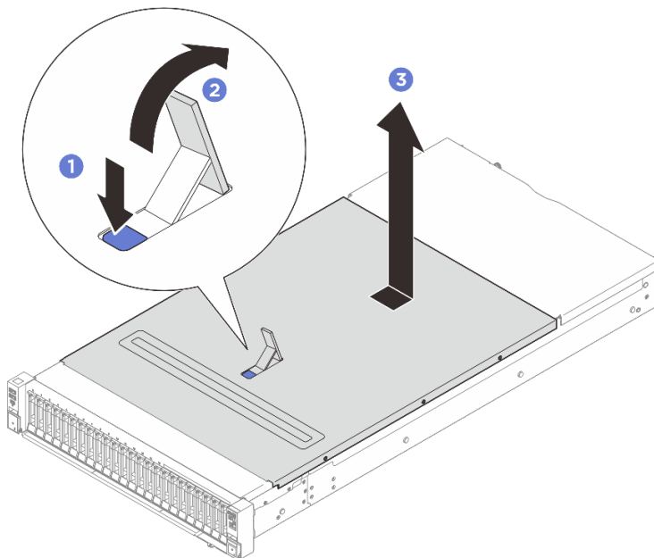
圖例 233. 卸下前方上蓋
