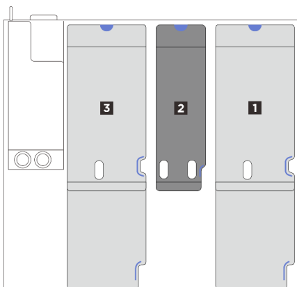
圖例 169. 配備三個 PCIe 擴充卡和擴充卡延伸器的伺服器型號
