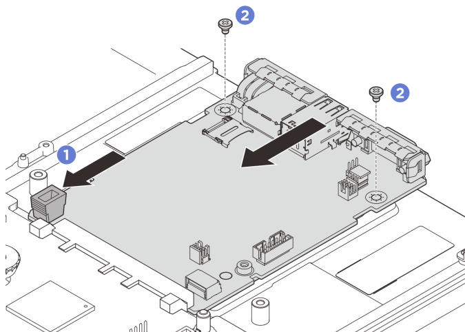
圖例 226. 安裝系統 I/O 板
