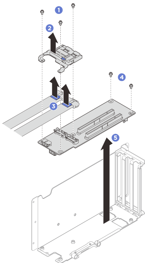
圖例 176. 卸下 PCIe 擴充卡
