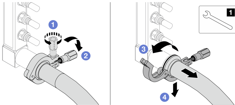
圖例 140. 將歧管與軟管套件分離
