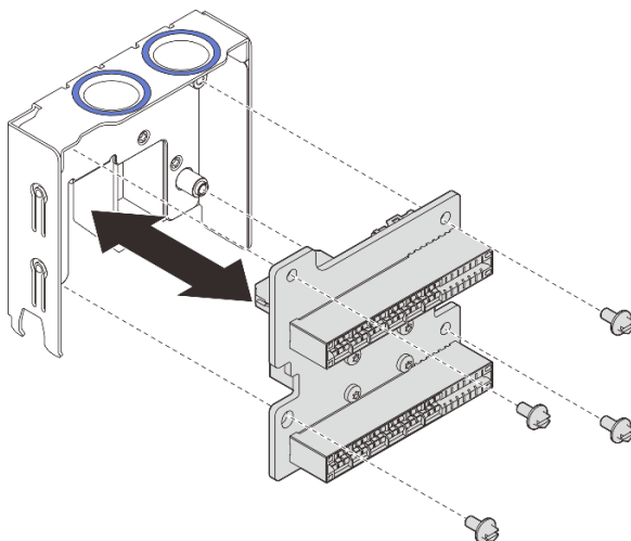
圖例 186. 拆卸電源配送板
