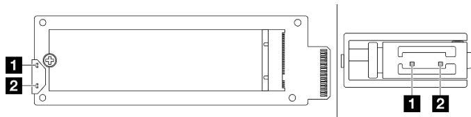
圖例 251. 背面 M.2 轉插卡 LED
