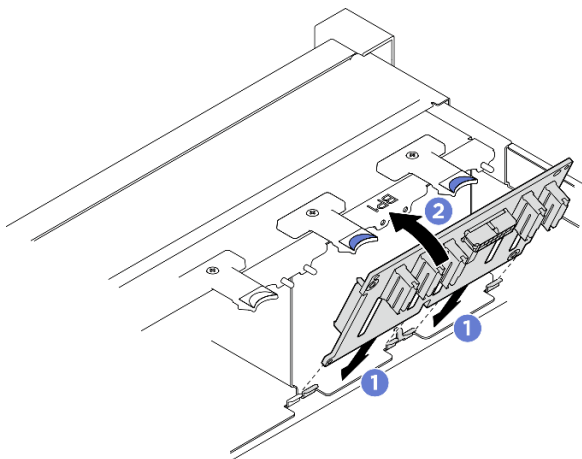
圖例 6. 安裝 2.5 吋硬碟背板
