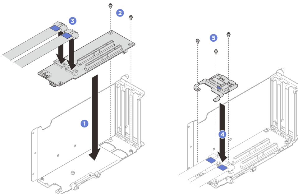
圖例 178. 安裝 PCIe 擴充卡
