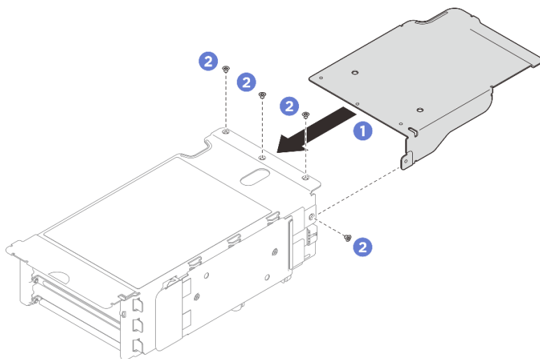
圖例 184. 安裝 PCIe 擴充卡延伸器
