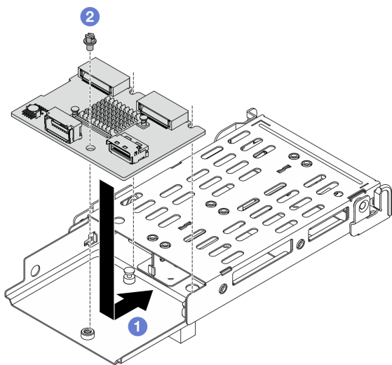
圖例 209. 安裝 M.2 開機配接卡
