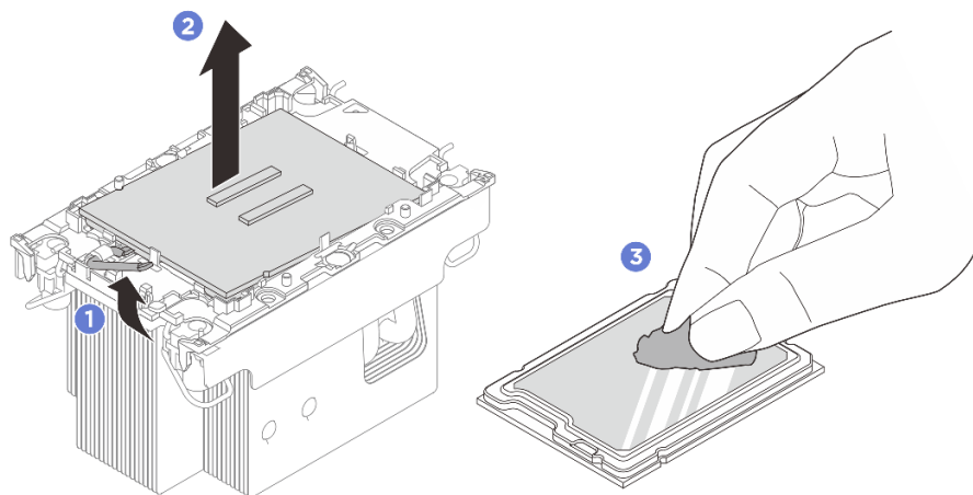
圖例 193. 將處理器與散熱槽和支架分開
