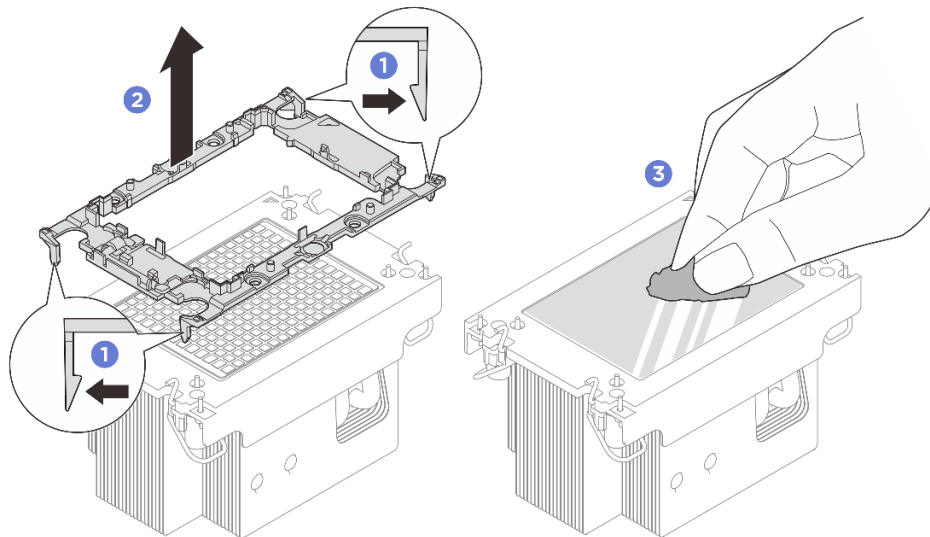
圖例 194. 將處理器支架與散熱槽分開
