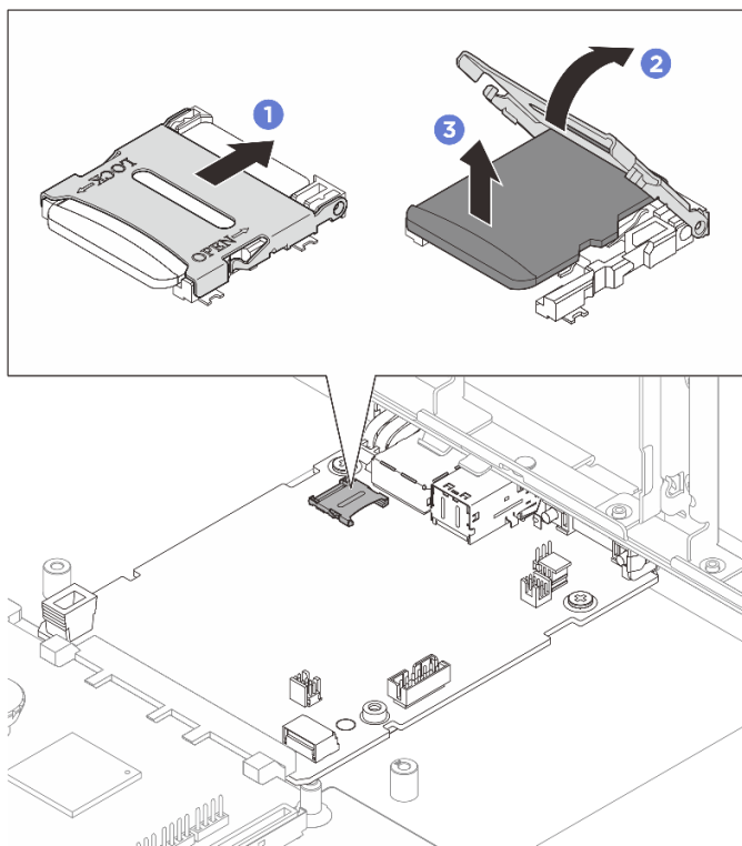
圖例 156. 卸下 MicroSD 卡
