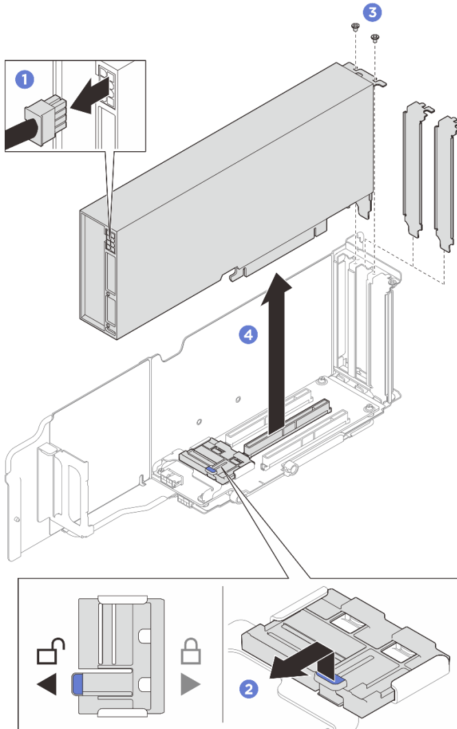
圖例 59. 卸下雙寬 GPU 配接卡
