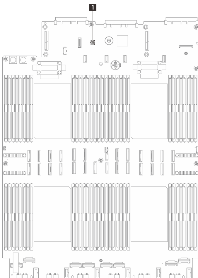
圖例 95. 連接洩漏偵測感應器模組
