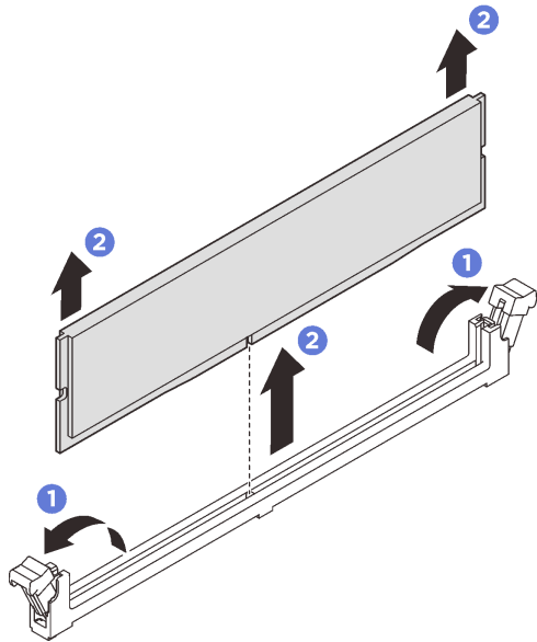
圖例 172. 卸下記憶體模組
