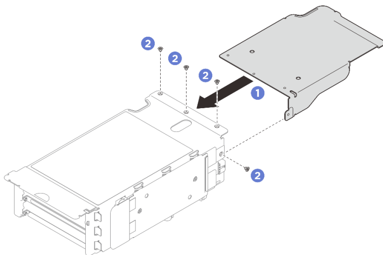
圖例 203. 安裝 PCIe 擴充卡延伸器
