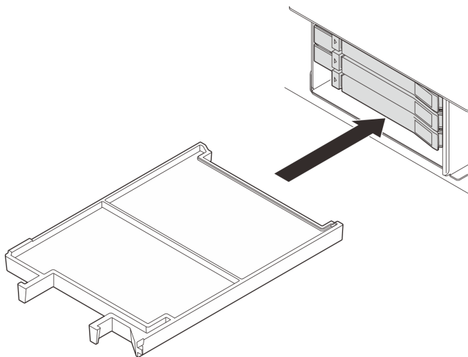
圖例 61. 安裝機槽填充板
