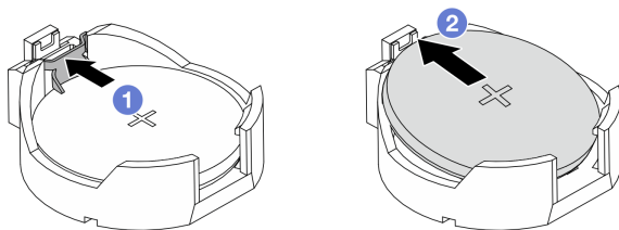
圖例 40. 取出 CMOS 電池
