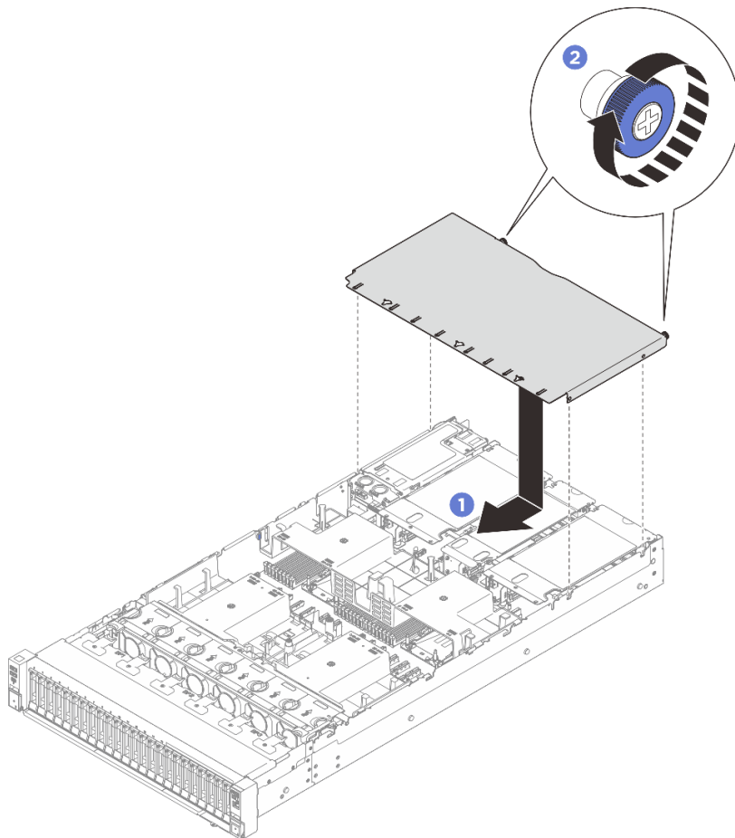
圖例 254. 安裝後方上蓋
