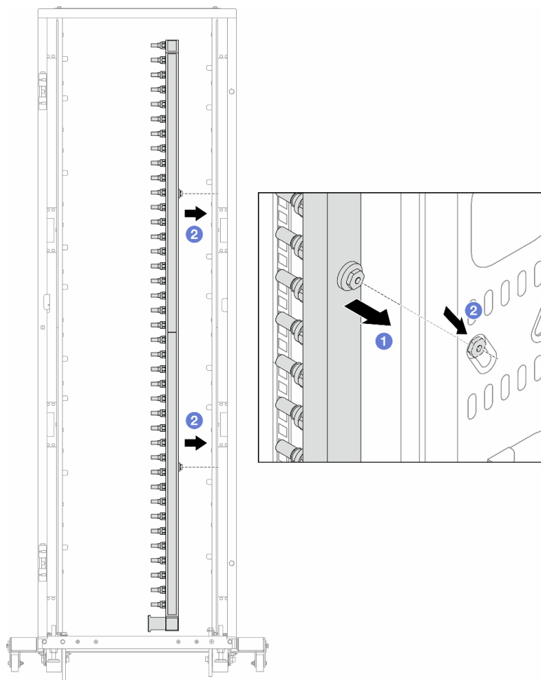
圖例 160. 安裝歧管
