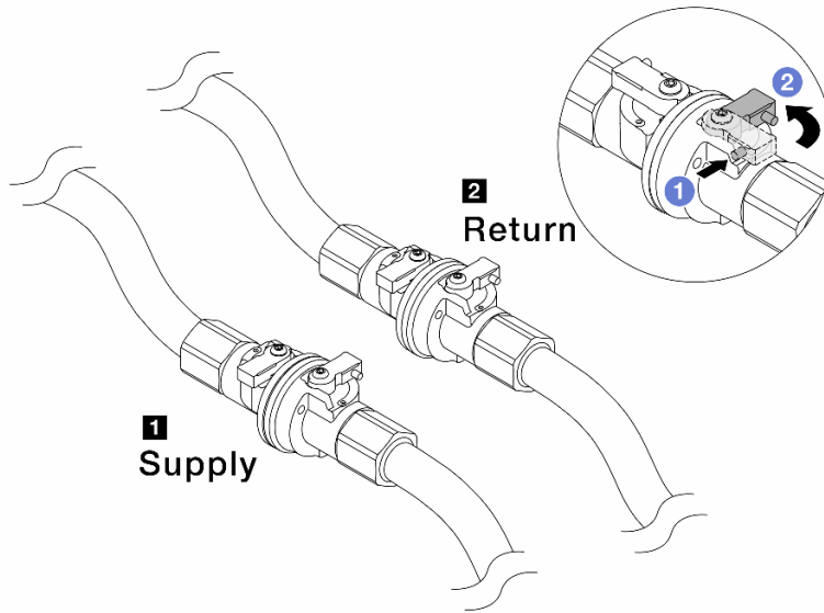
圖例 152. 關閉球閥
