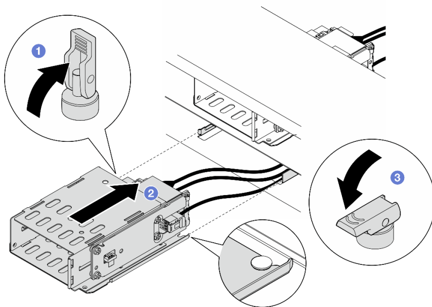
圖例 55. 安裝 E3.S 2T 框架
