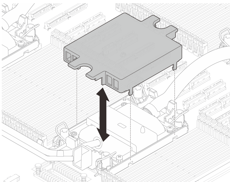
圖例 98. 卸下水冷板蓋
