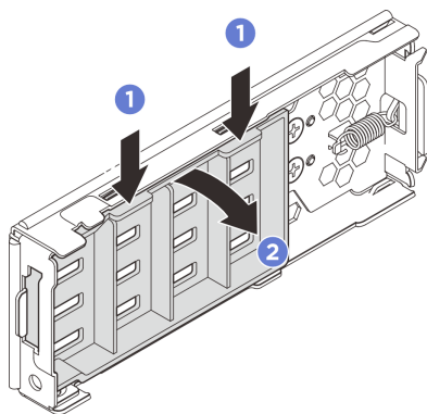
圖例 62. 卸下內板
