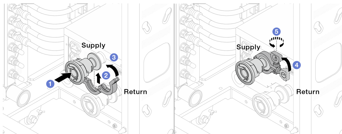
圖例 140. 安裝球閥
