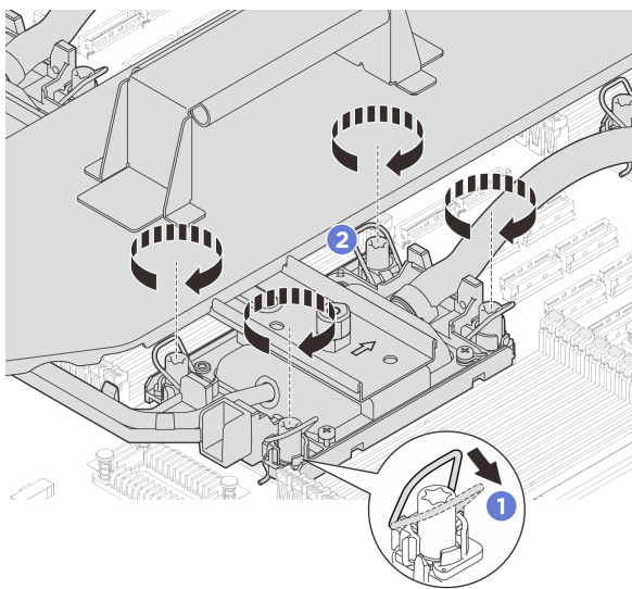
圖例 109. 鎖緊 Torx T30 螺帽
