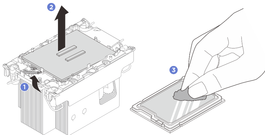
圖例 212. 將處理器與散熱槽和支架分開
