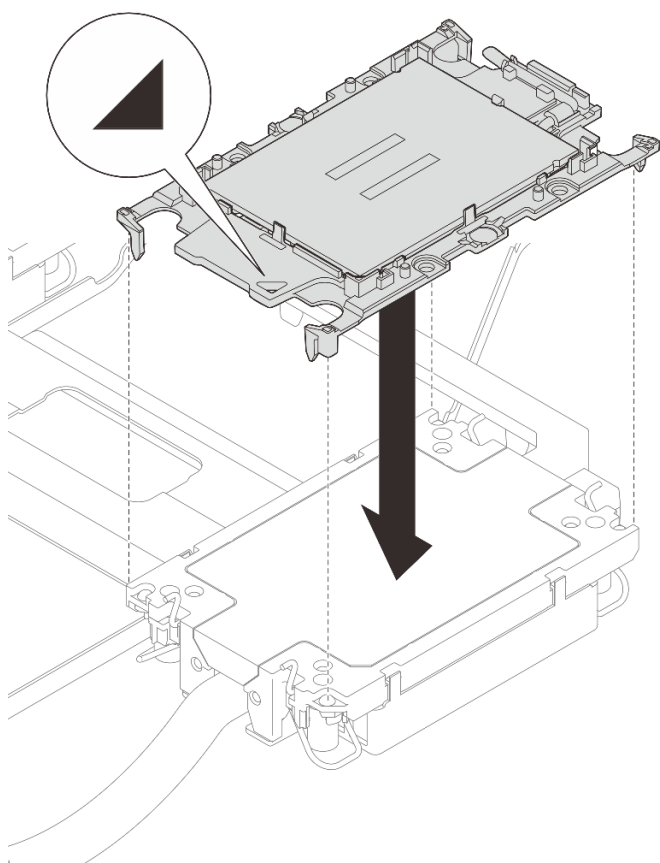
圖例 106. 將處理器安裝到水冷板
