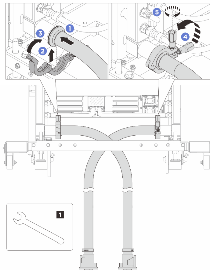
圖例 162. 安裝水管套件
