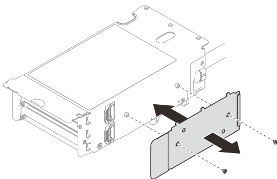
圖例 196. 卸下纜線蓋
