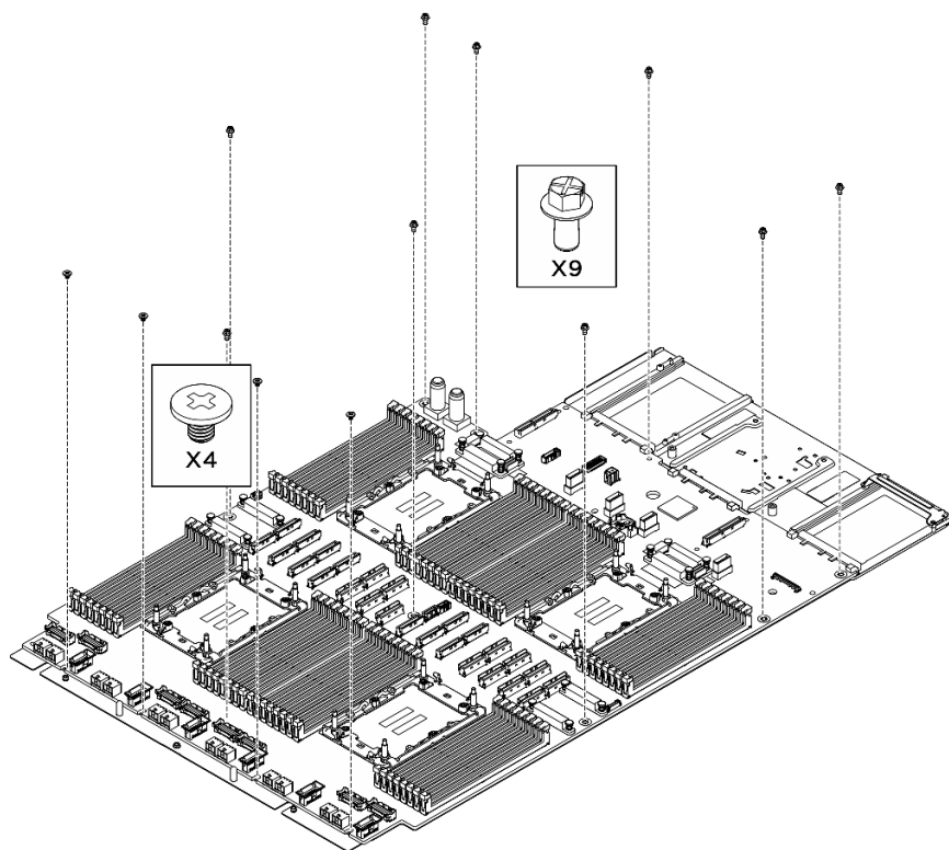
圖例 279. 卸下螺絲
