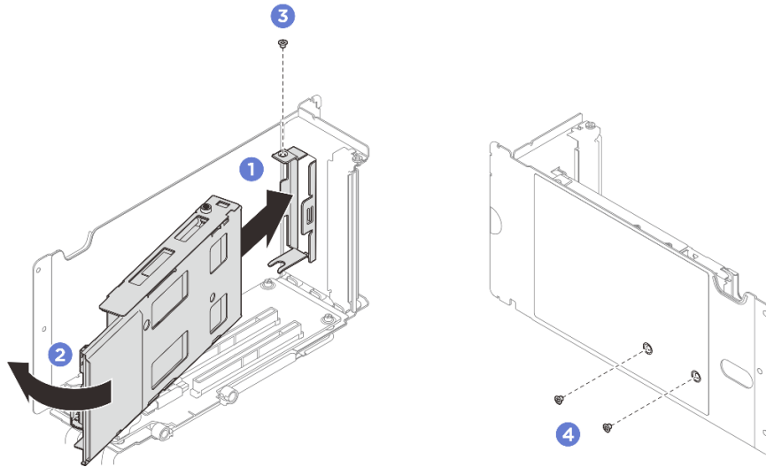
圖例 229. 安裝 M.2 框架
