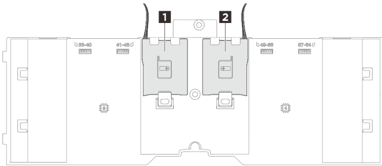
圖例 74. 快閃記憶體電源模組插槽位置
