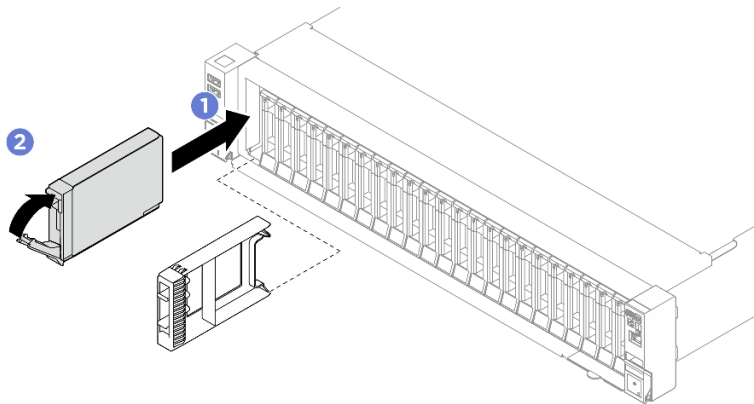
圖例 26. 安裝 2.5 吋熱抽換硬碟
