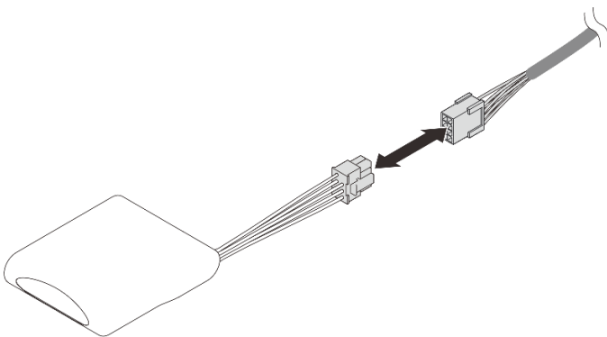
圖例 38. 連接快閃記憶體電源模組纜線
