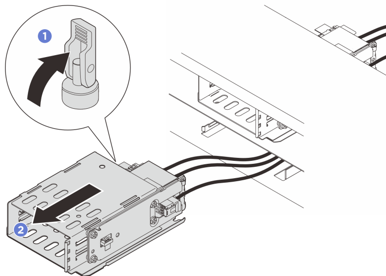
圖例 64. 卸下 E3.S 1T 框架
