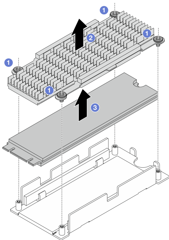
圖例 86. 將 M.2 硬碟和散熱槽分開
