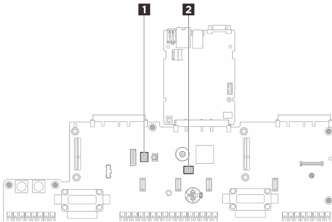
圖例 15. 主機板組件開關
