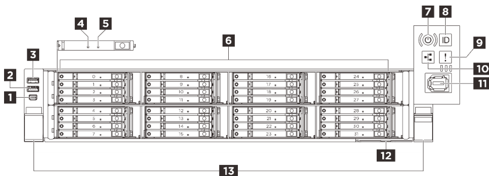
圖例 3. 配備 E3.S 1T 機槽之伺服器型號的正面圖
