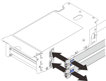
圖例 194. 拔除纜線
