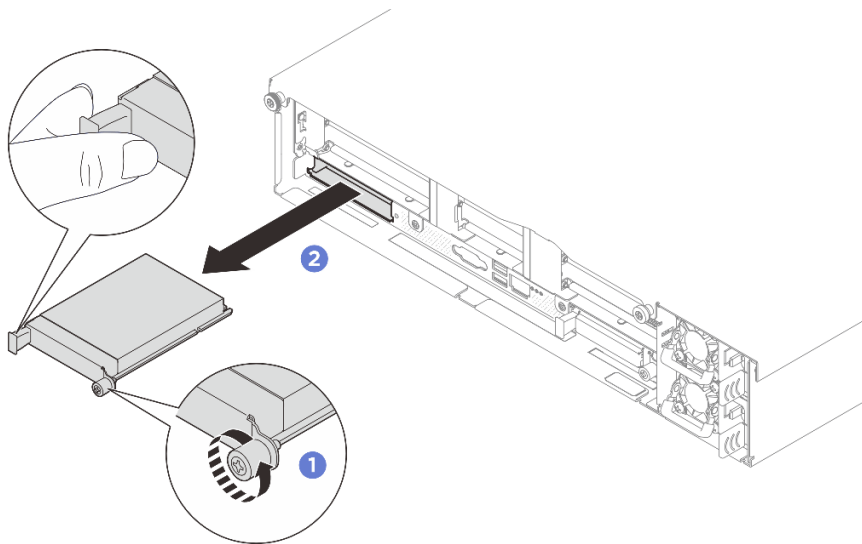
圖例 177. 卸下 OCP 模組
