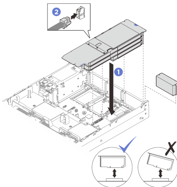
圖例 192. 安裝 PCIe FHFL 擴充卡
