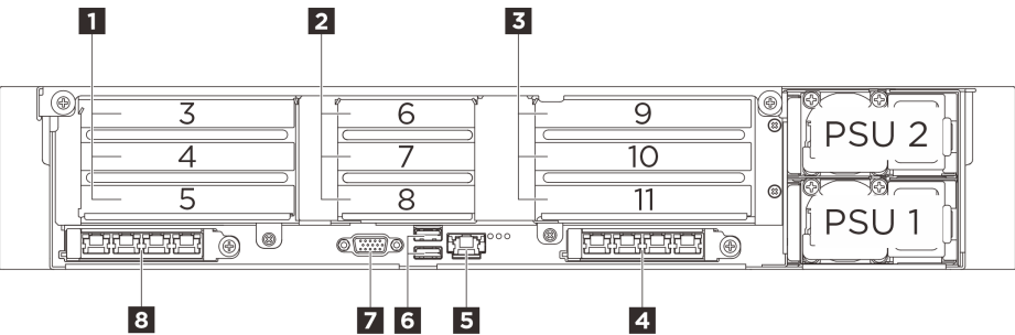
圖例 5. 配備三個 PCIe 擴充卡之伺服器型號的背面圖
