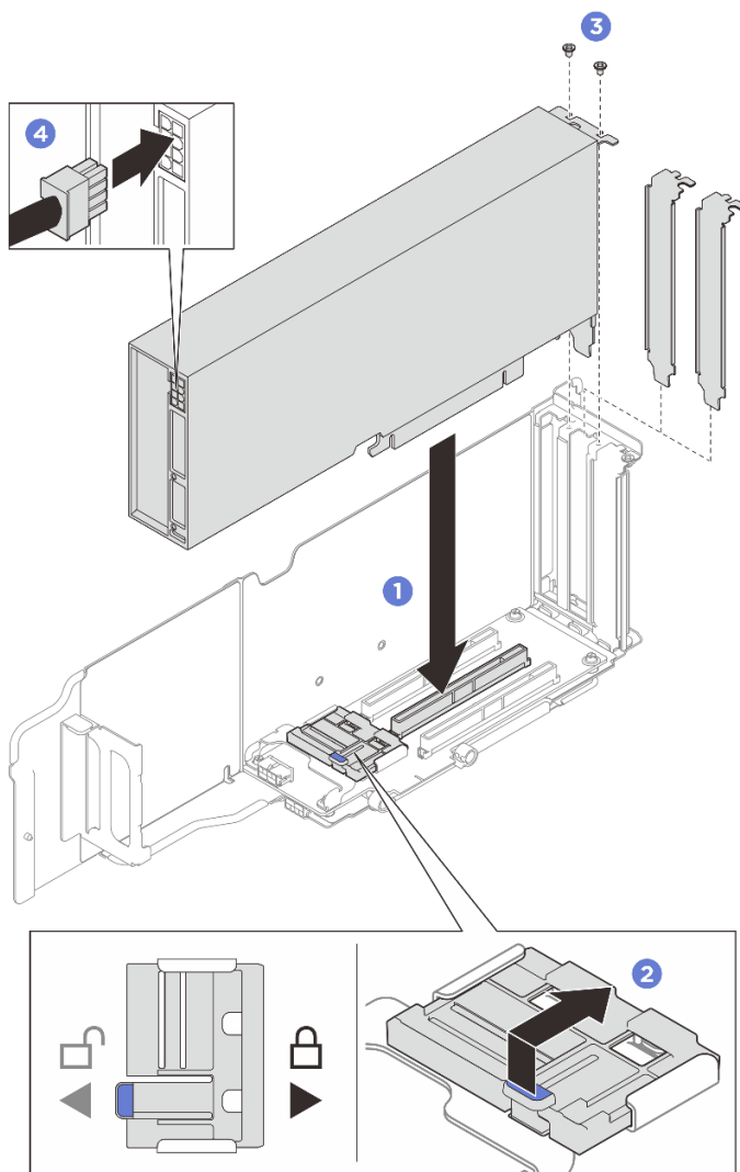
圖例 80. 安裝雙寬 GPU 配接卡
