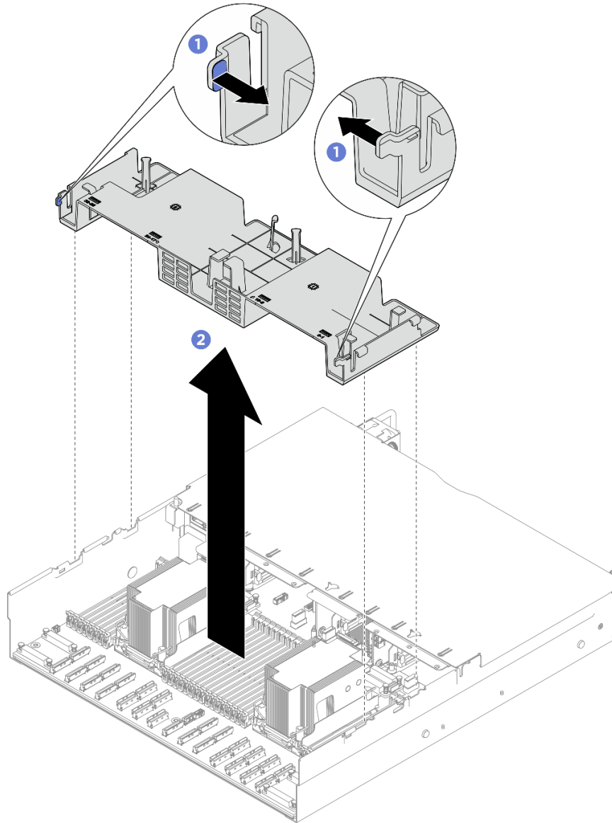
圖例 35. 卸下後方空氣擋板
