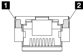
圖例 274. XCC 系統管理埠 (10/100/1000 Mbps RJ-45) 上的 LED
