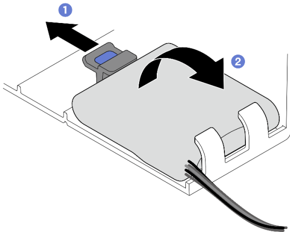
圖例 73. 卸下快閃記憶體電源模組
