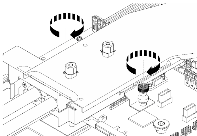
圖例 108. 安裝水冷板組件
