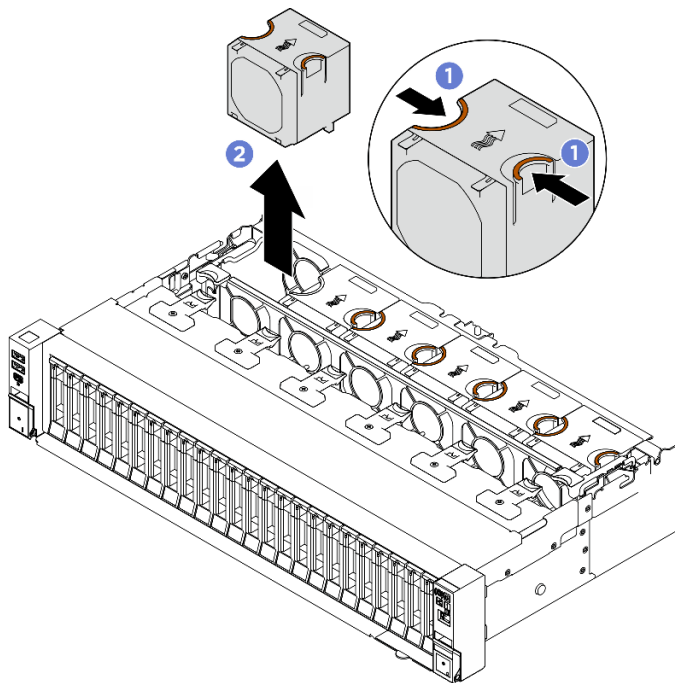
圖例 68. 卸下風扇
