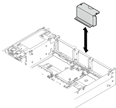
圖例 97. 卸下擴充卡填充板
