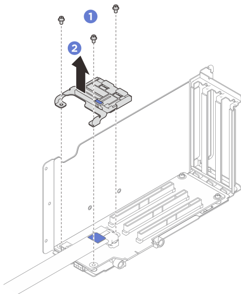
圖例 200. 卸下 PCIe 固定器
