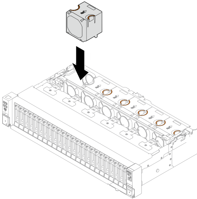
圖例 71. 安裝風扇
