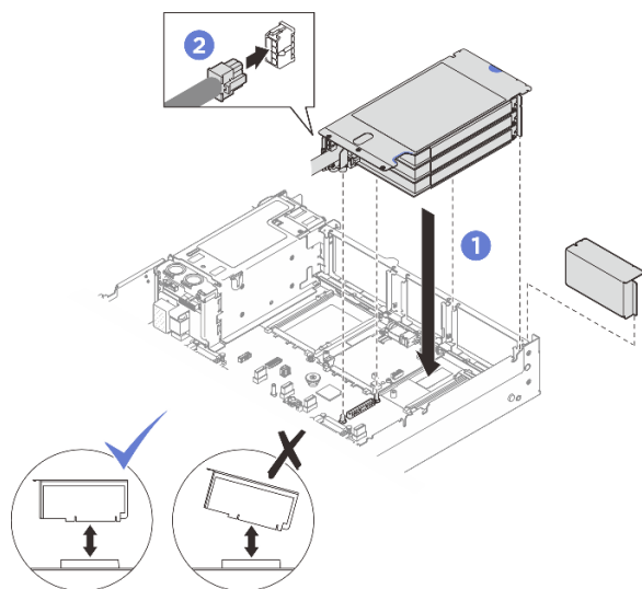
圖例 191. 安裝 PCIe FHHL 擴充卡
