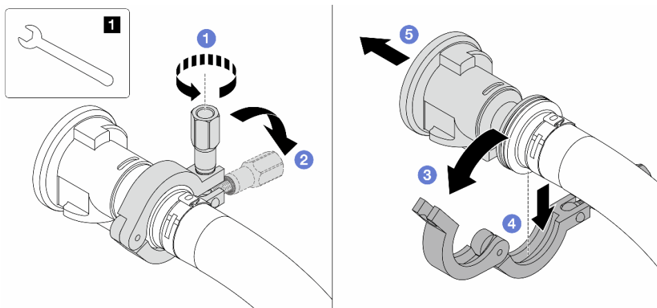
圖例 139. 分開球閥
