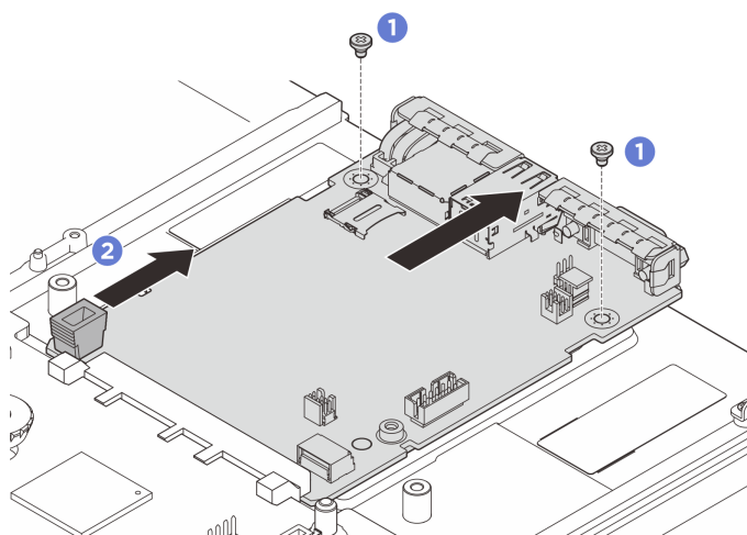
圖例 244. 卸下系統 I/O 板
