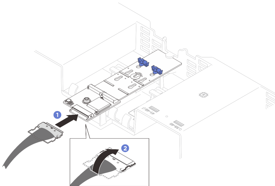
圖例 119. M.2 開機配接卡纜線連接方式
