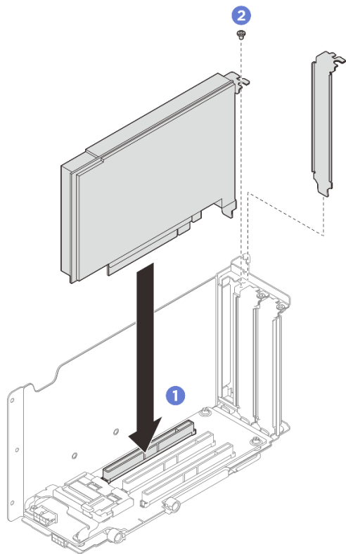
圖例 186. PCIe 配接卡安裝
