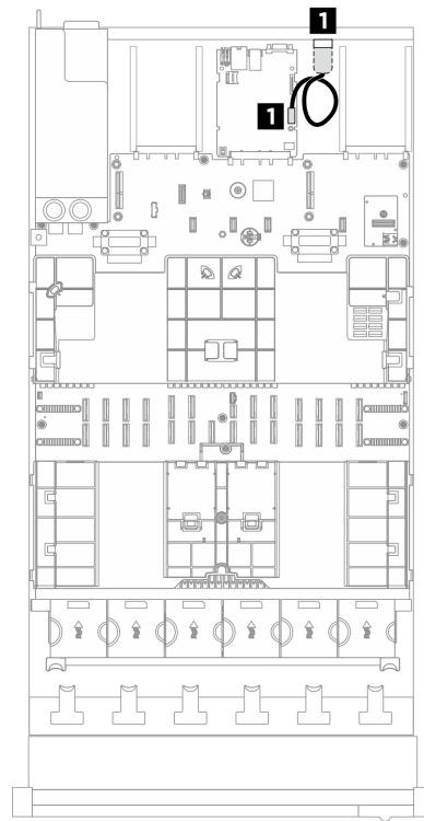
圖例 241. 配備四個 PCIe 擴充卡的伺服器型號的序列埠模組纜線佈線
