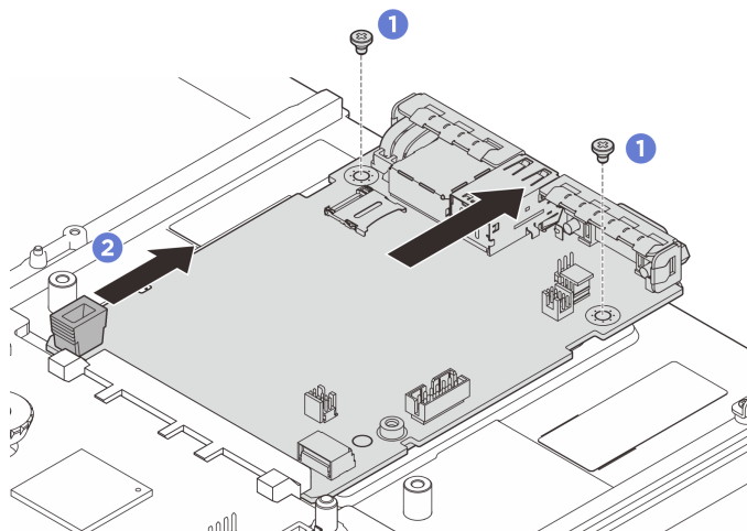
圖例 277. 卸下系統 I/O 板
