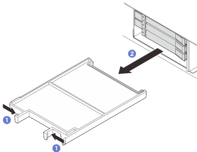
圖例 59. 卸下機槽填充板
