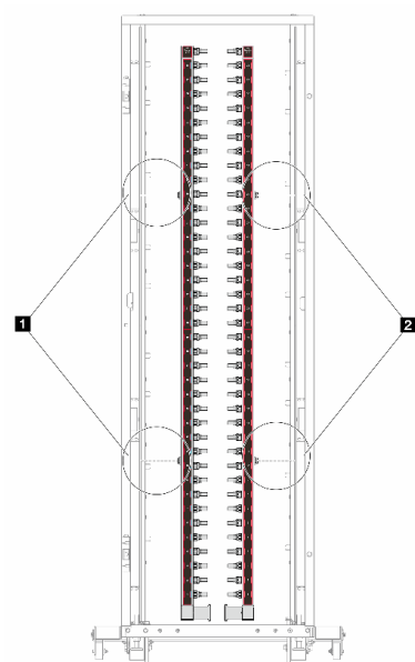
圖例 123. 42U 排式系統中的歧管
