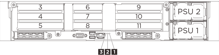
圖例 271. 背面系統 LED
