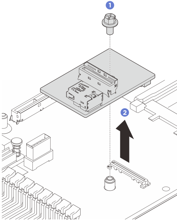
圖例 257. 卸下 USB I/O 板
