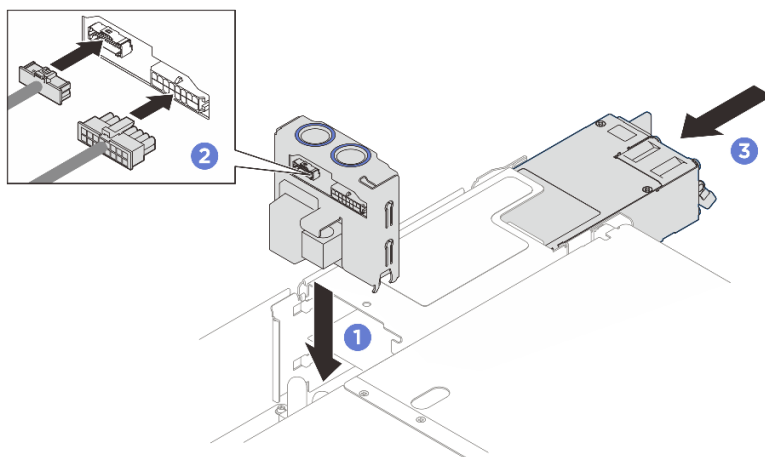
圖例 206. 安裝電源配送板
