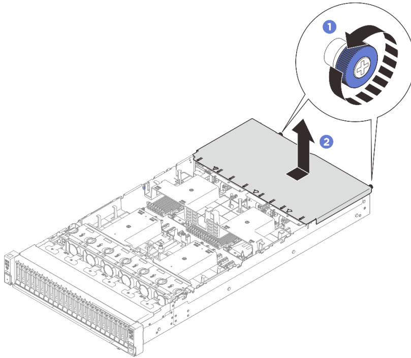
圖例 253. 卸下後方上蓋
