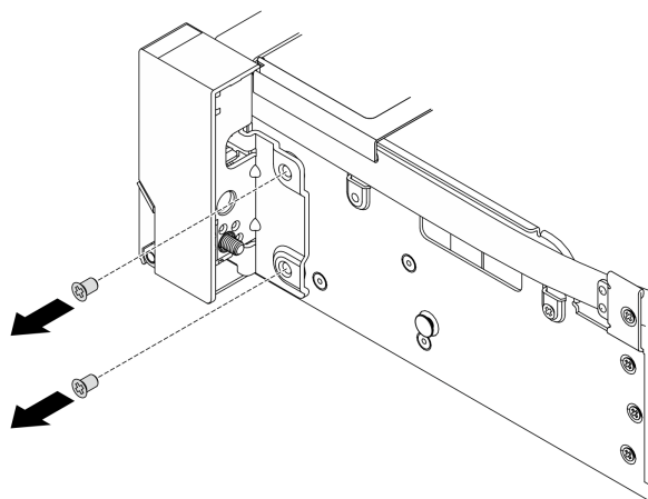
圖例 221. 卸下螺絲
