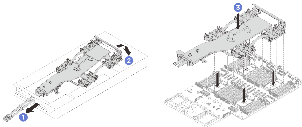
圖例 107. 安裝水冷板組件
