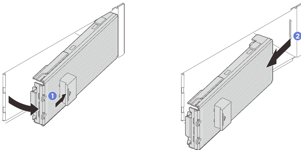
圖例 43. 卸下 E3.S 擋板
