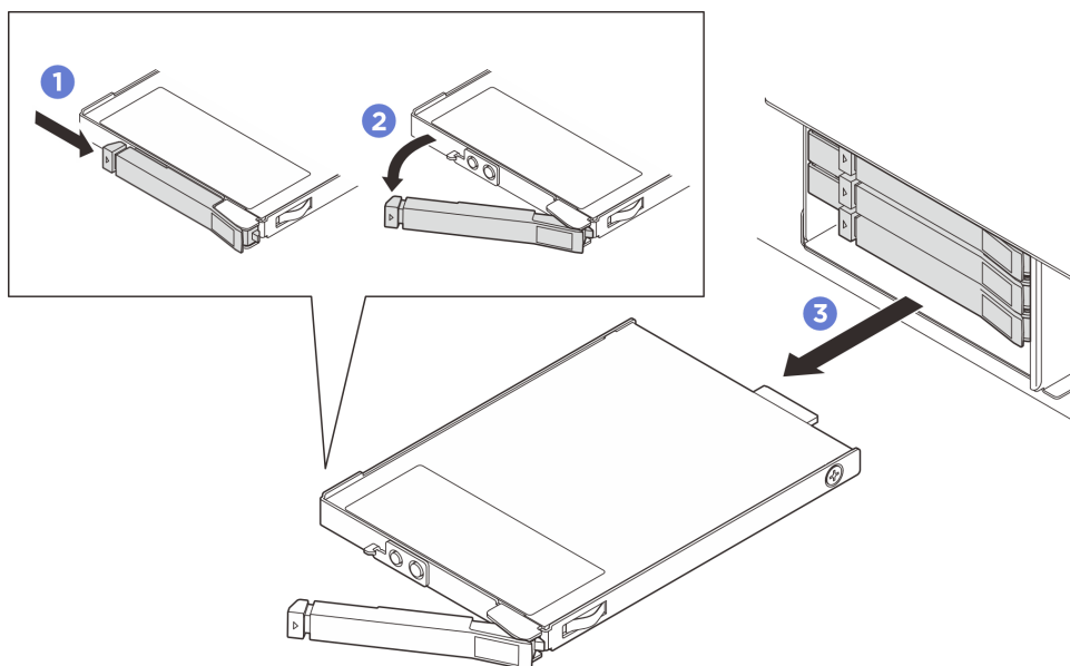
圖例 57. 卸下 E3.S 熱抽換硬碟
