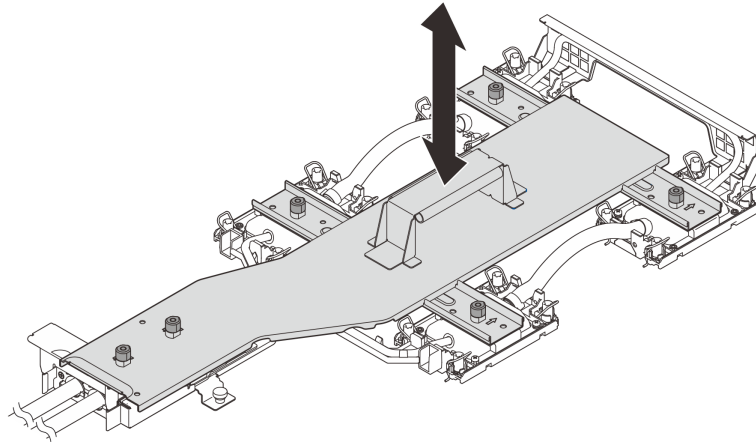
圖例 99. 安裝水冷板支架
