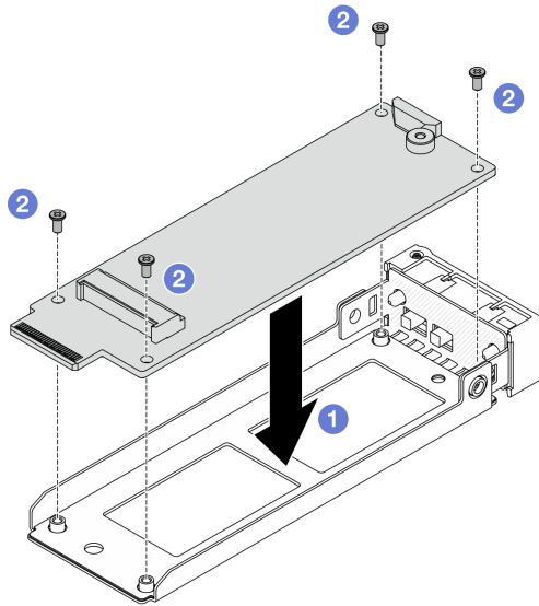
圖例 90. 安裝 M.2 轉插卡
