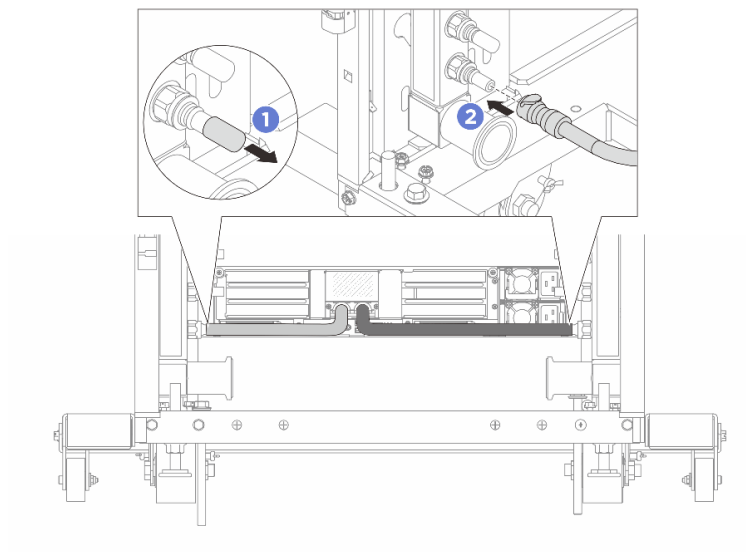
圖例 161. 安裝快速連接插件
