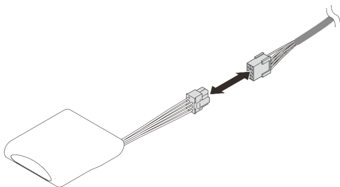
圖例 27. 拔掉快閃記憶體電源模組纜線
