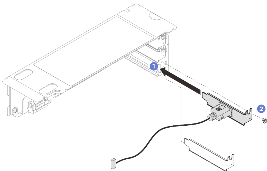
圖例 238. 序列埠模組安裝
