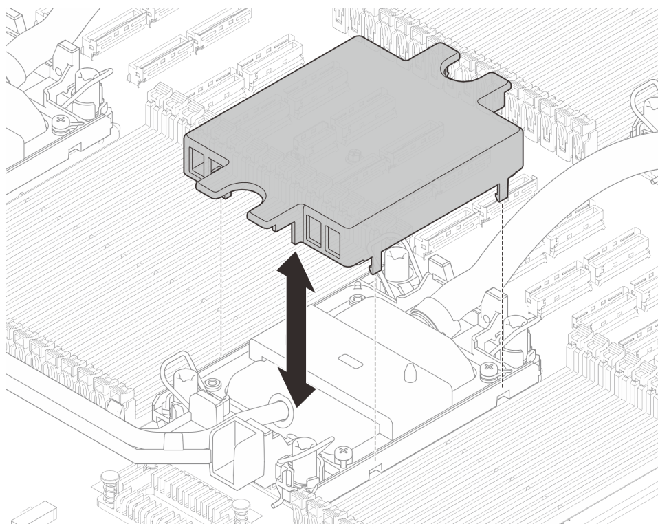
圖例 276. 拆下水冷板蓋
