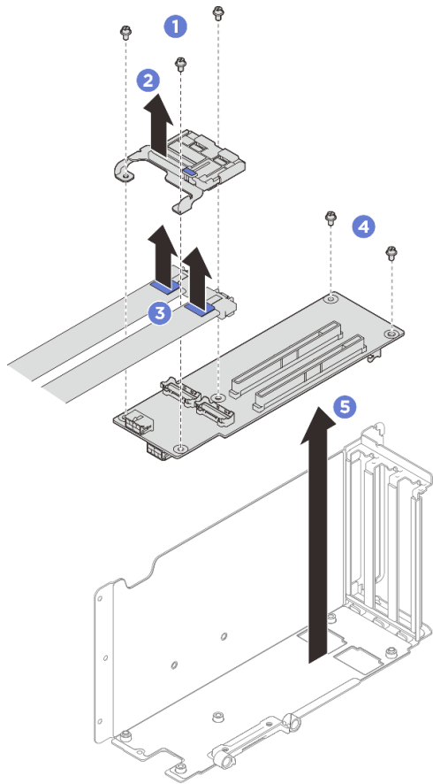
圖例 195. 卸下 PCIe 擴充卡
