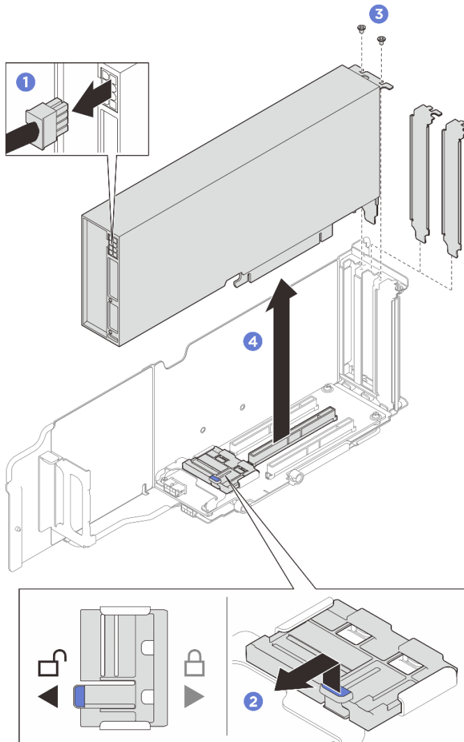
圖例 78. 卸下雙寬 GPU 配接卡
