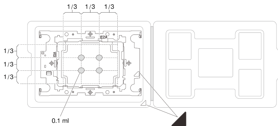
圖例 216. 運送匣中的處理器塗上散熱膏
