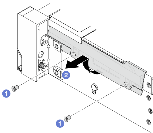
圖例 220. 卸下纜線固定夾
