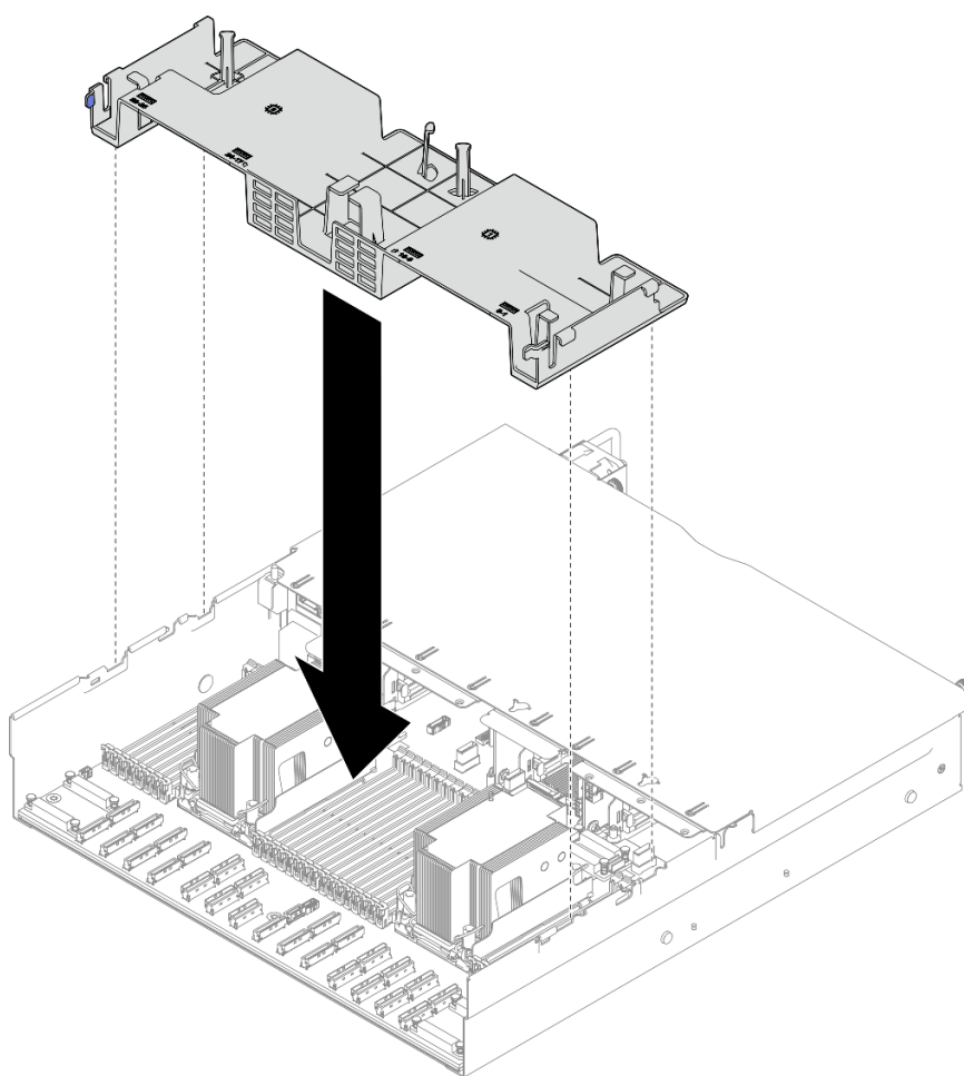
圖例 36. 安裝後方空氣擋板
