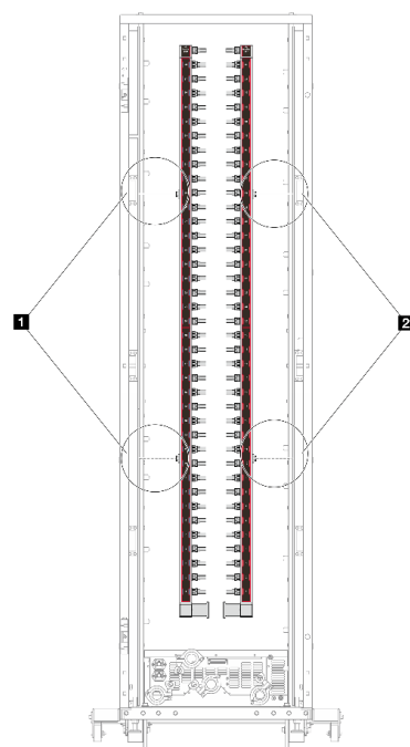
圖例 125. 48U 機架式系統中的歧管
