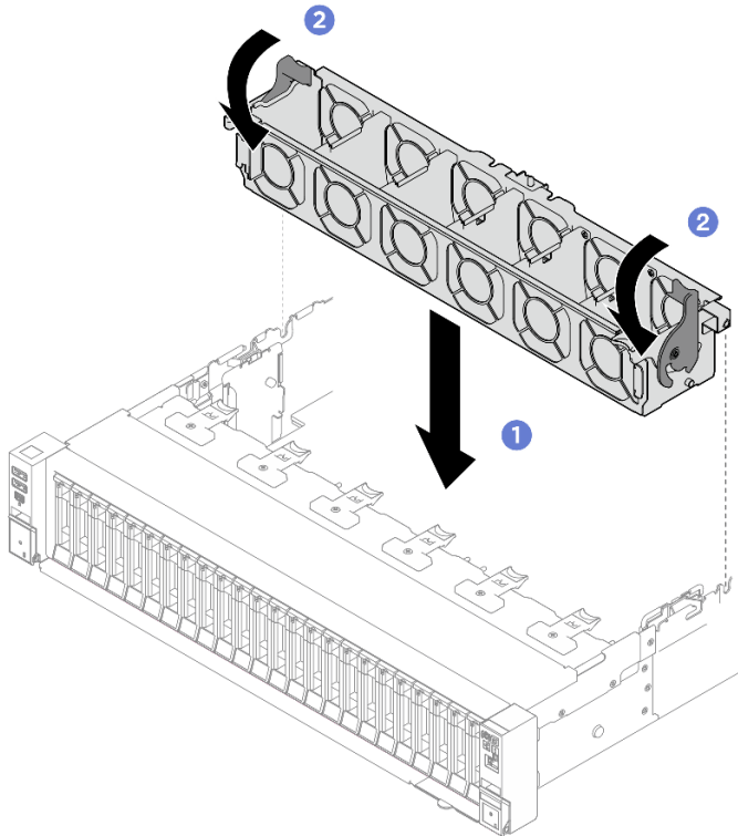
圖例 70. 安裝風扇機盒
