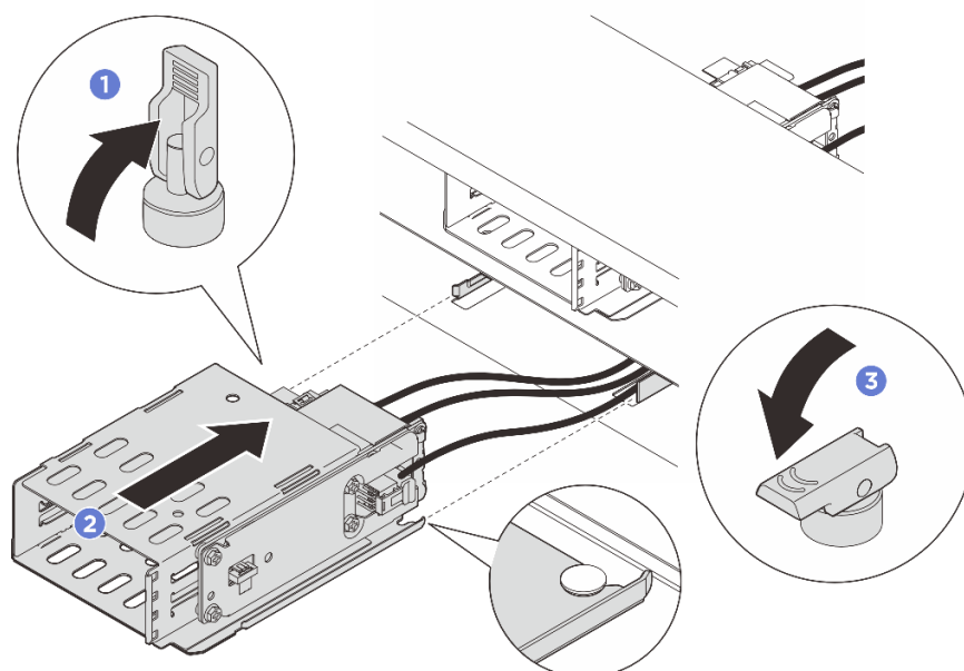
圖例 67. 安裝 E3.S 1T 框架
