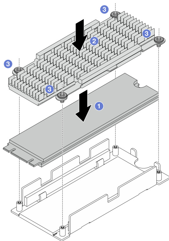
圖例 89. 組裝散熱槽和 M.2 硬碟
