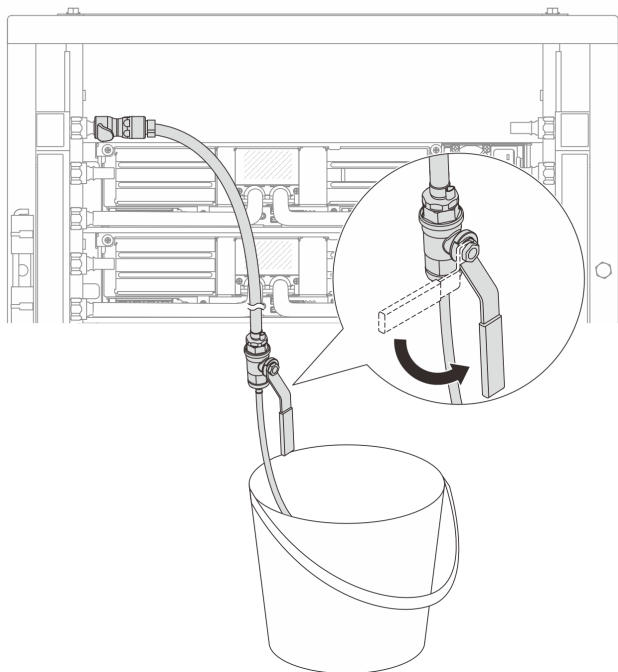
圖例 169. 開啟供應側的洩放閥門
