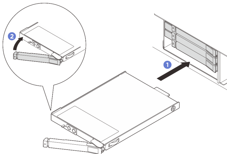
圖例 60. 安裝 E3.S 熱抽換硬碟
