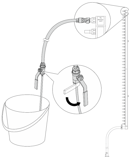
圖例 158. 開啟洩放閥門
