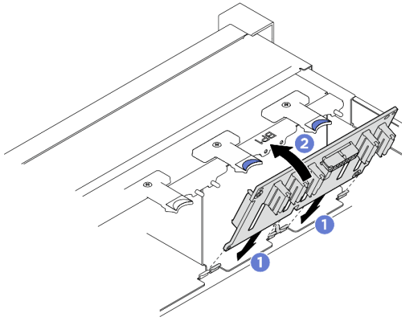
圖例 25. 安裝 2.5 吋硬碟背板
