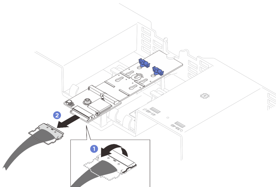
圖例 28. 拔除 M.2 開機配接卡纜線
