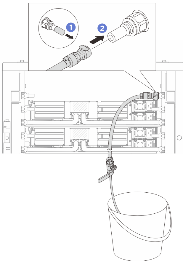
圖例 166. 在回流側安裝洩放套件
