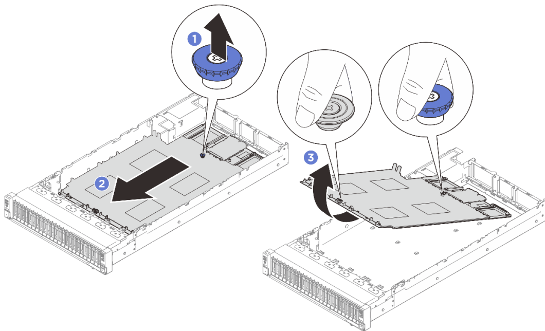
圖例 247. 卸下主機板組件
