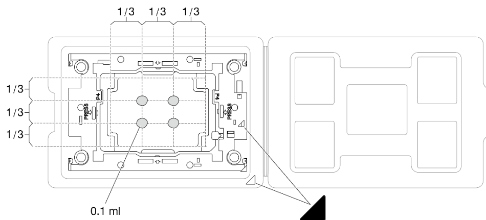
圖例 105. 運送匣中的處理器塗上散熱膏
