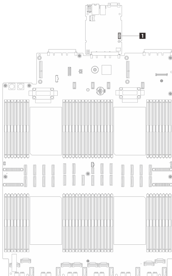
圖例 239. 序列埠接頭位置
