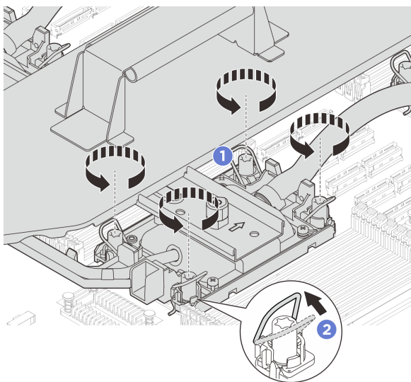
圖例 101. 鬆開 Torx T30 螺帽
