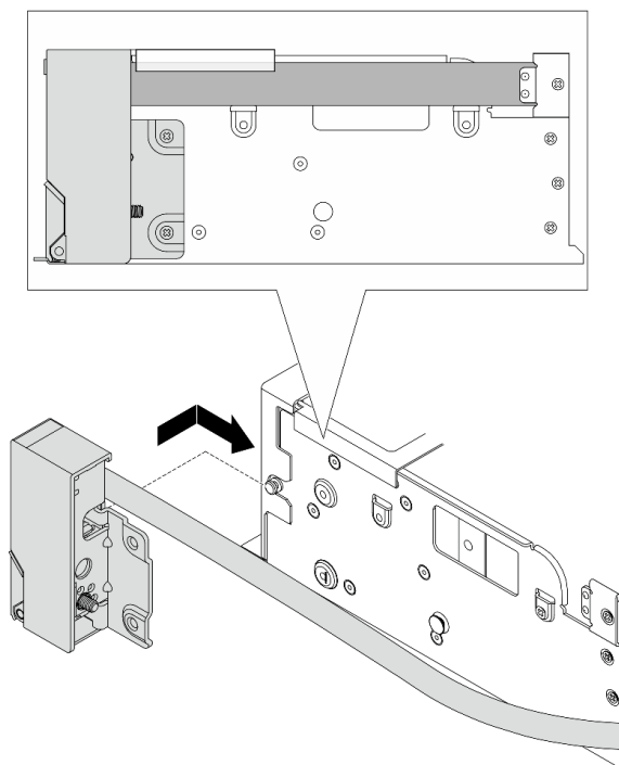
圖例 223. 安裝機架門鎖
