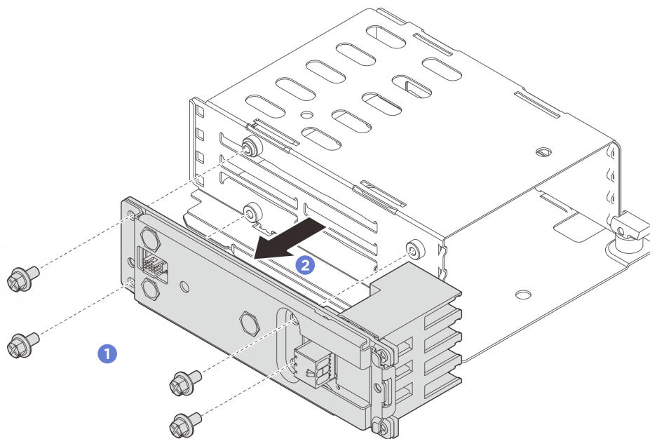
圖例 65. 卸下背板組件
