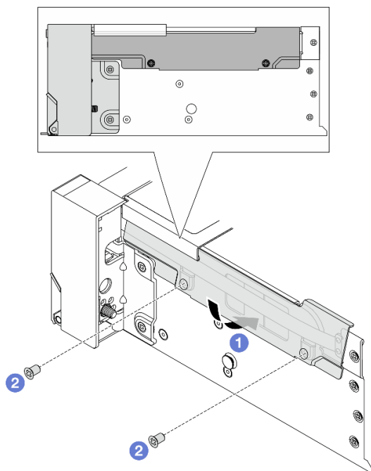
圖例 225. 安裝纜線固定夾
