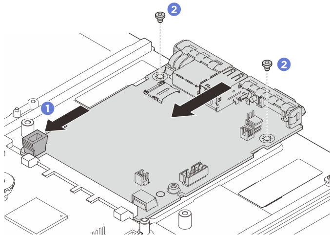
圖例 249. 安裝系統 I/O 板
