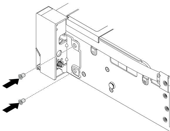
圖例 224. 鎖上螺絲
