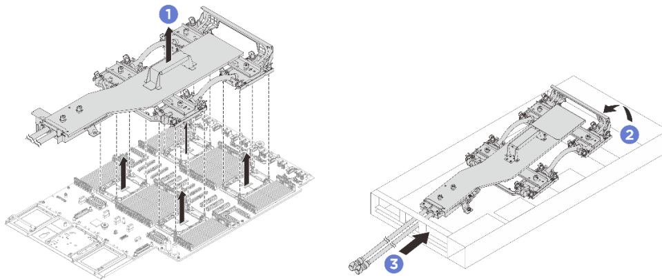
圖例 103. 卸下水冷板組件
