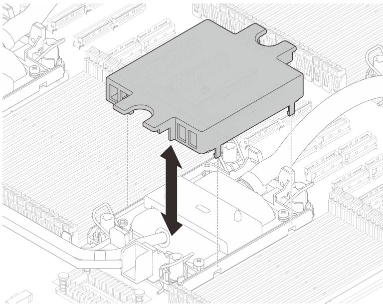
圖例 112. 安裝水冷板蓋
