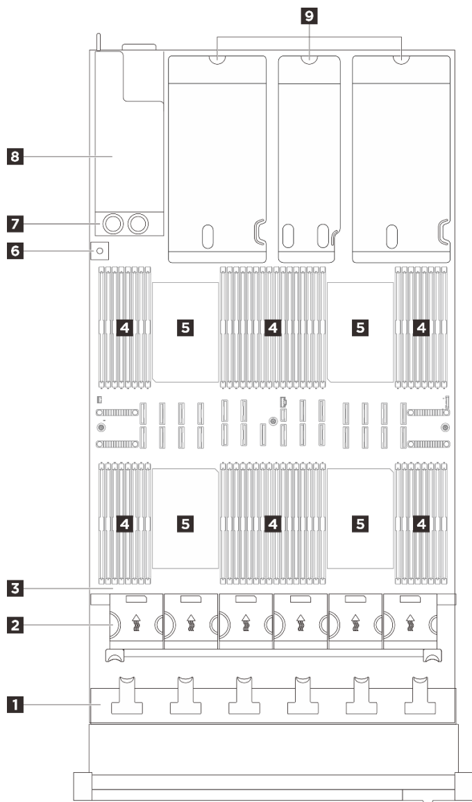
圖例 11. 配備三個 PCIe 擴充卡之伺服器型號的俯視圖
