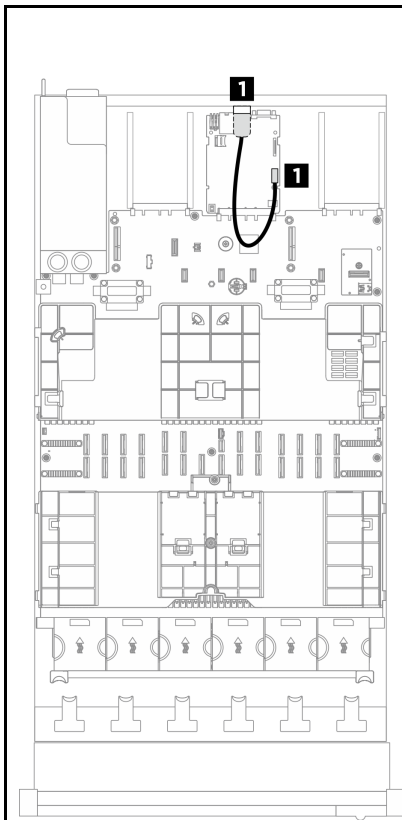
圖例 240. 配備三個 PCIe 擴充卡的伺服器型號的序列埠模組纜線佈線
