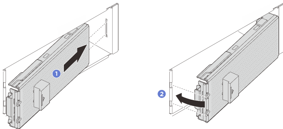
圖例 51. 安裝 E3.S 擋板
