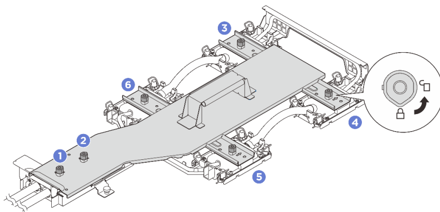
圖例 110. 鬆開水冷板支架
