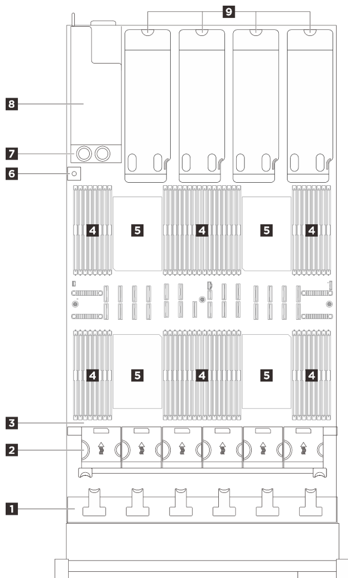
圖例 12. 配備四個 PCIe 擴充卡之伺服器型號的俯視圖
