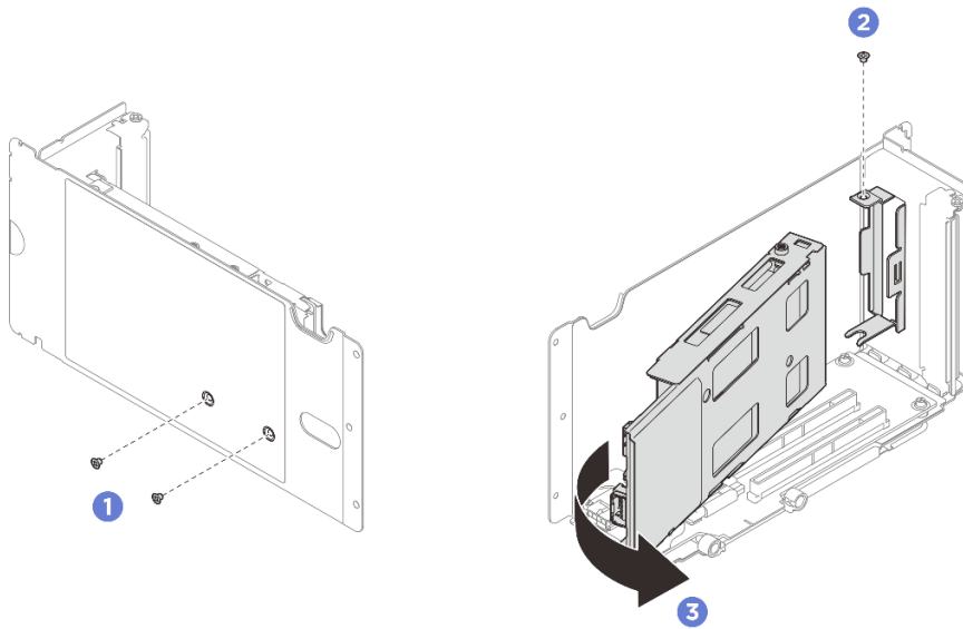
圖例 226. 卸下 M.2 框架
