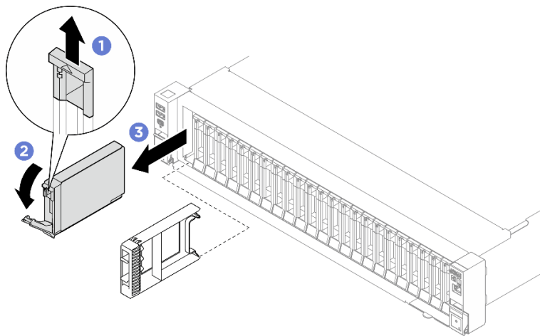
圖例 23. 卸下 2.5 吋熱抽換硬碟
