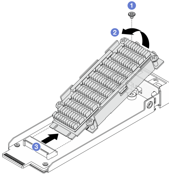
圖例 84. 卸下帶有散熱槽的 M.2 硬碟
