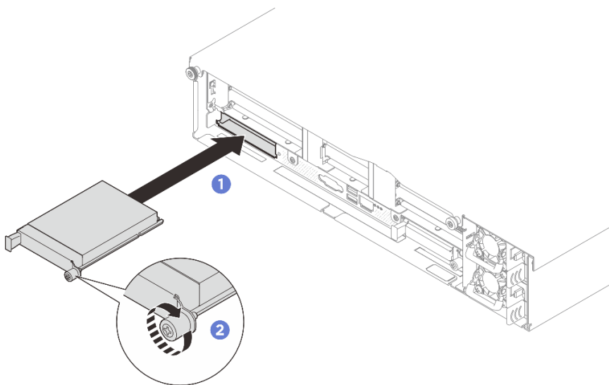
圖例 178. OCP 模組安裝
