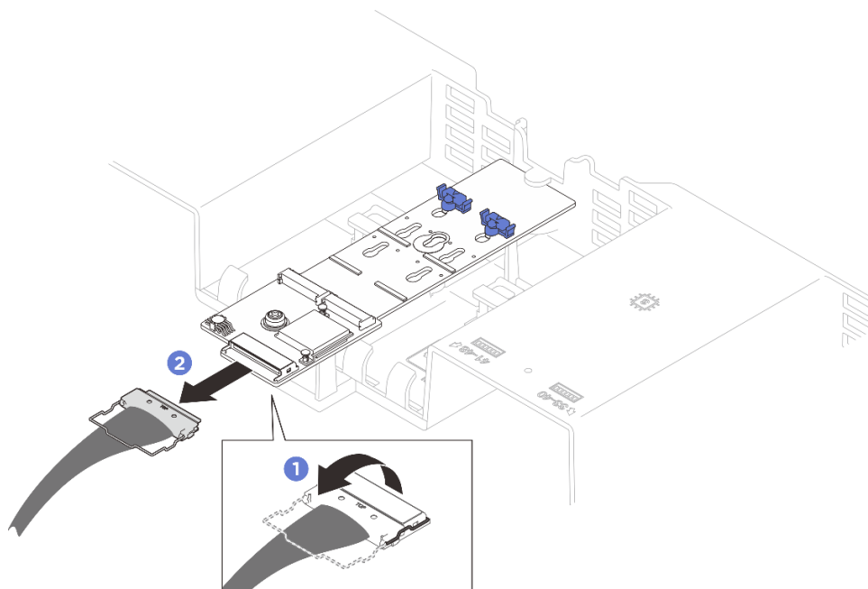
圖例 34. 拔除 M.2 開機配接卡纜線
