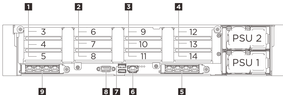
圖例 8. 配備四個 PCIe 擴充卡之伺服器型號的背面圖
