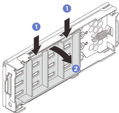
圖例 50. 卸下內板
