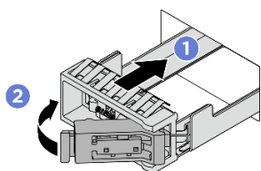
圖例 83. 安裝 M.2 硬碟匣
