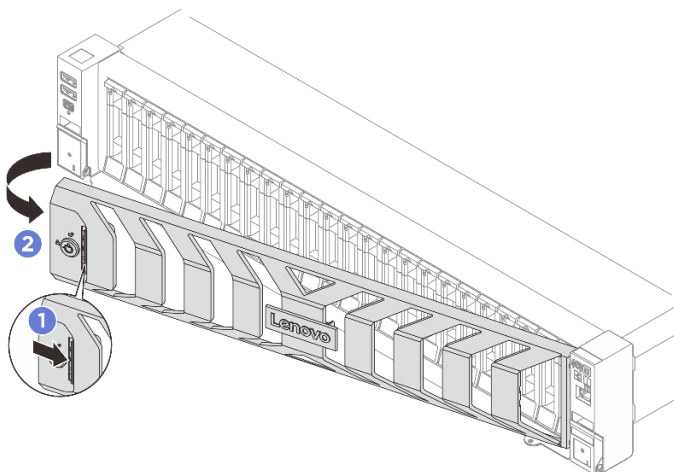
圖例 233. 卸下安全擋板
