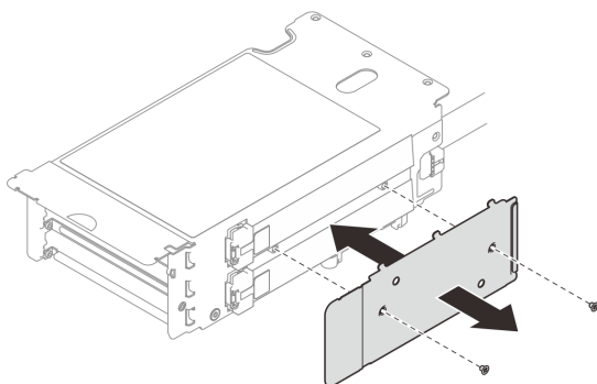
圖例 193. 卸下纜線蓋
