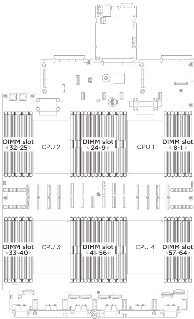
圖例 171. 記憶體模組和處理器佈置
