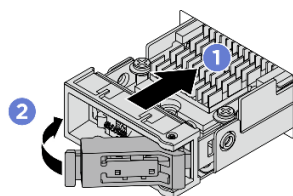
圖例 93. 安裝 M.2 硬碟組件
