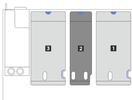
圖例 179. 配備三個 PCIe 擴充卡的伺服器型號
