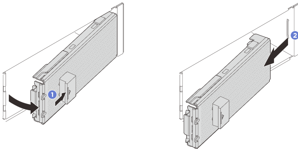
圖例 58. 卸下 E3.S 擋板
