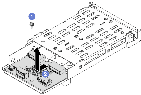
圖例 227. 卸下 M.2 開機配接卡
