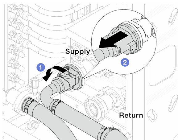
圖例 131. 卸下連接套組
