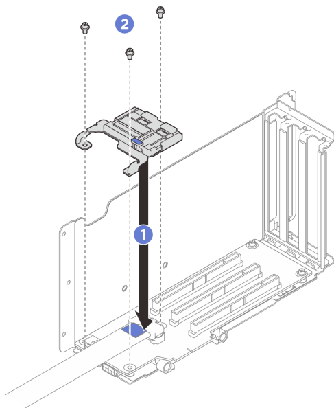
圖例 201. 安裝 PCIe 固定器
