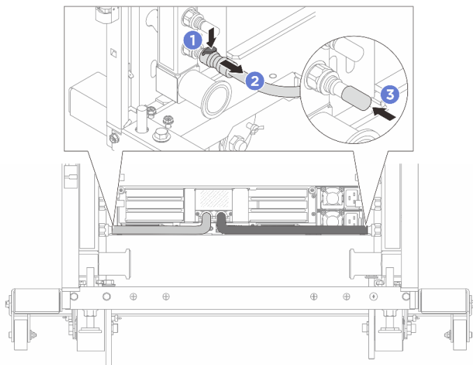
圖例 153. 移除 quick connect 插頭
