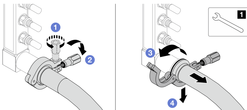
圖例 159. 將歧管與軟管套件分離
