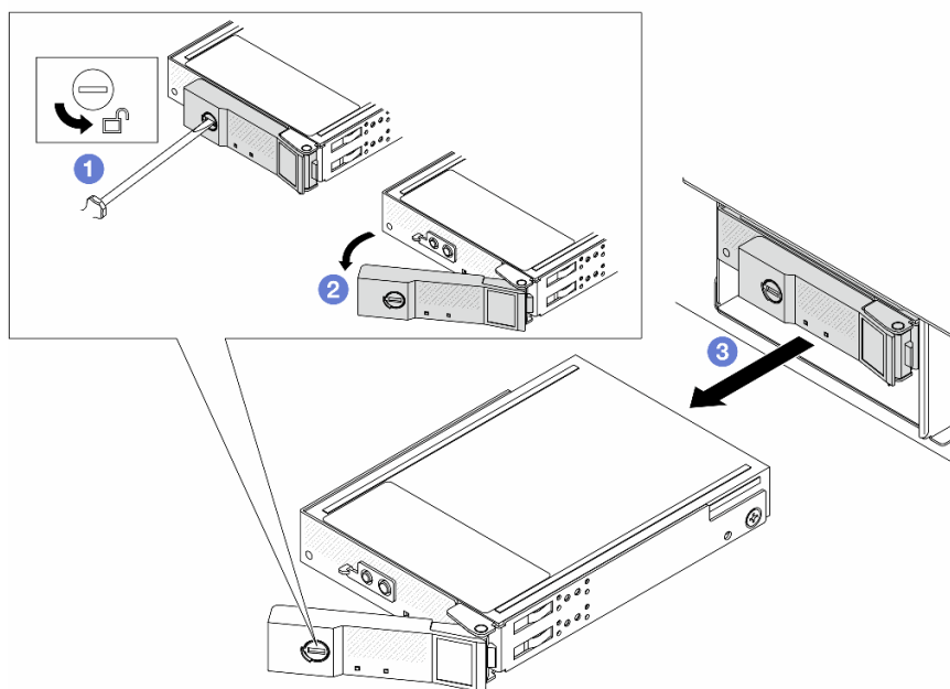
圖例 44. 卸下 CMM
