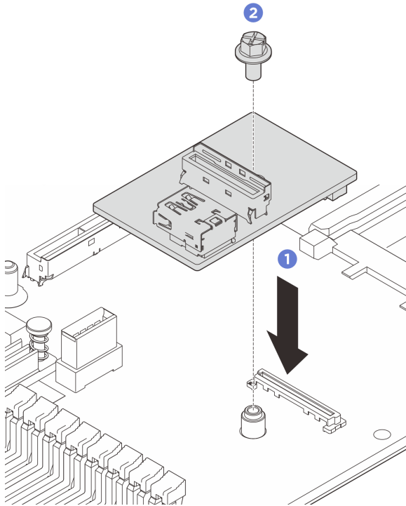
圖例 258. 安裝 USB I/O 板
