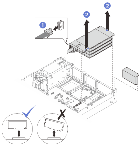
圖例 183. 卸下 PCIe FHFL 擴充卡
