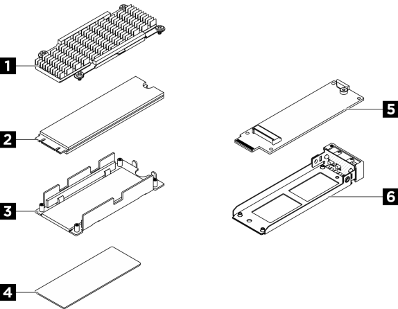
圖例 81. 熱抽換 M.2 硬碟組件的零件
