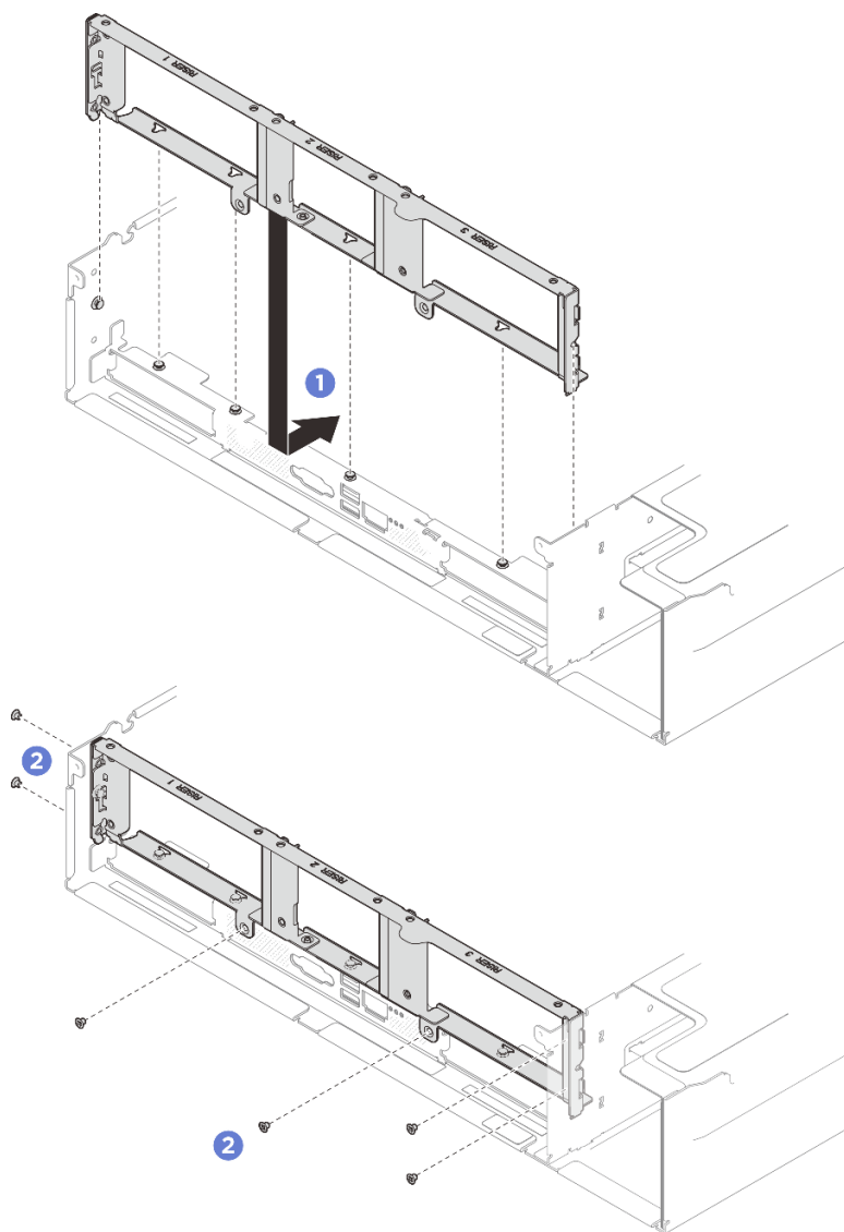
圖例 231. 後壁安裝
