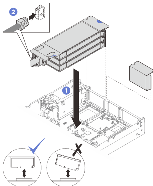
圖例 190. 安裝 PCIe LP 擴充卡 (含電源線)
