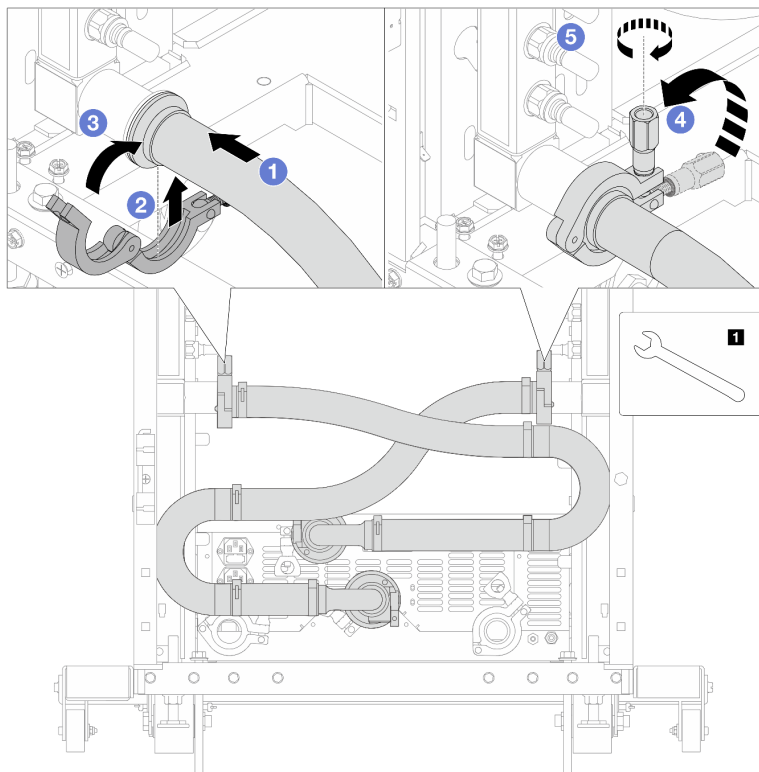
圖例 141. 安裝連接套組
