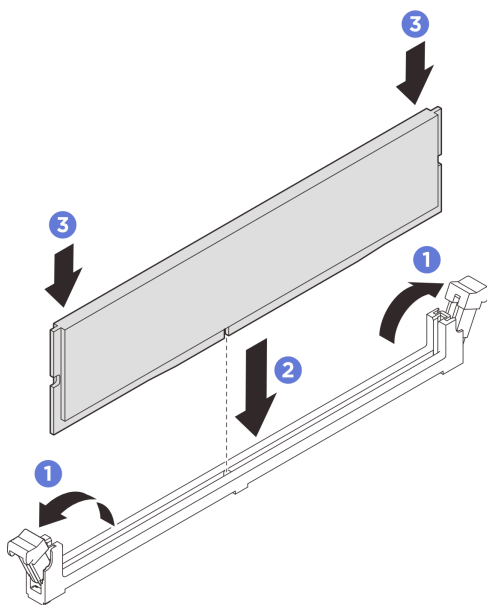
圖例 174. 安裝記憶體模組
