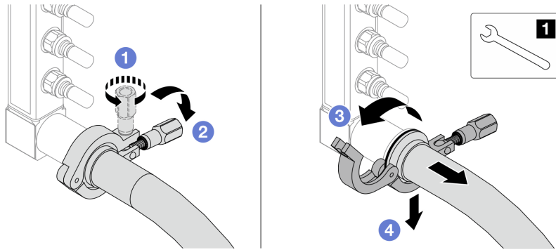
圖例 137. 將歧管與連接套組分開
