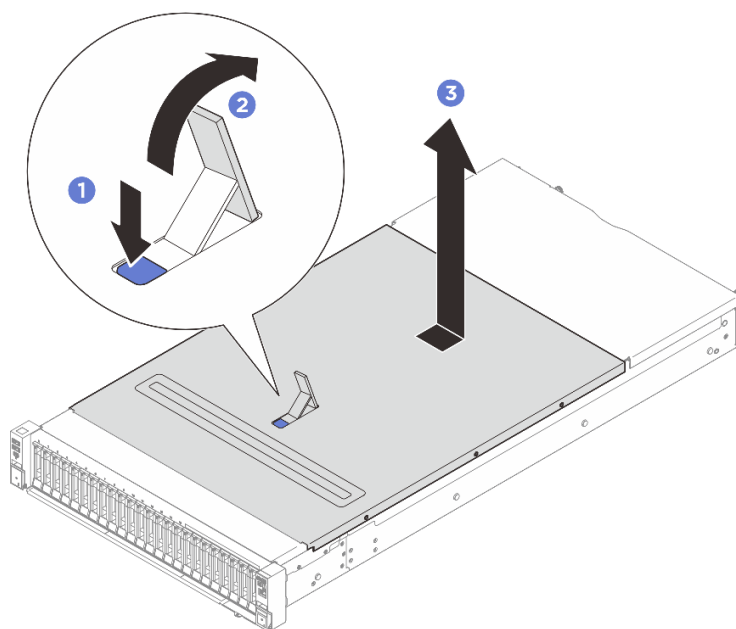
圖例 252. 卸下前方上蓋
