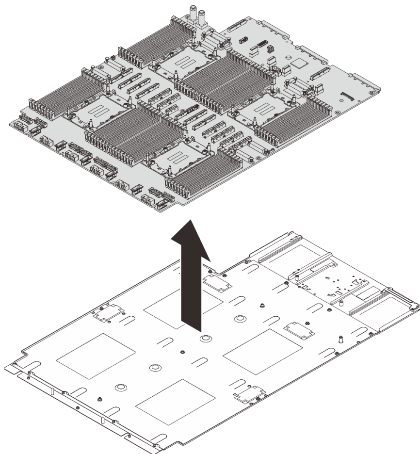
圖例 280. 拆卸處理器板
