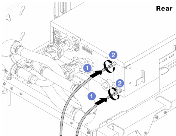
圖例 144. CDU 的背面
