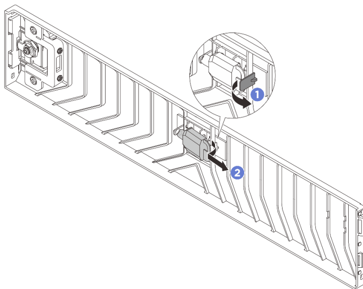
圖例 234. 取出鑰匙
