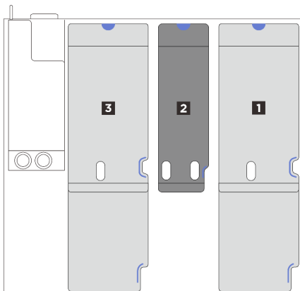
圖例 188. 配備三個 PCIe 擴充卡和擴充卡延伸器的伺服器型號
