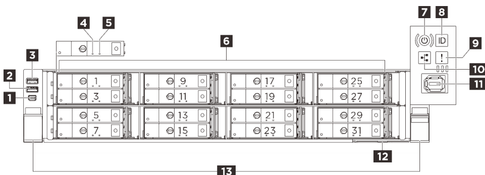
圖例 4. 配備 E3.S 2T 機槽之伺服器型號的正面圖
