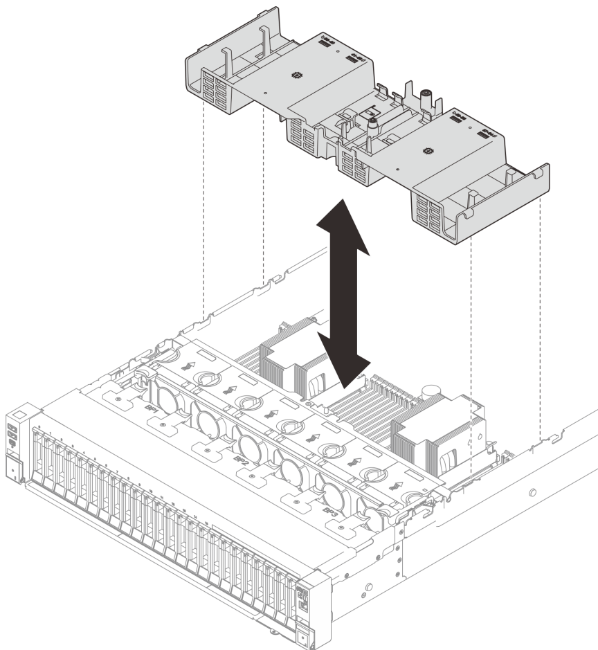
圖例 30. 安裝前方空氣擋板
