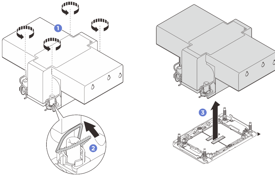
圖例211. 卸下 2U 效能 PHM
