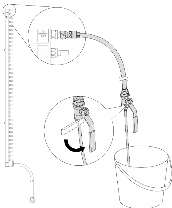
圖例 156. 開啟洩放閥門
