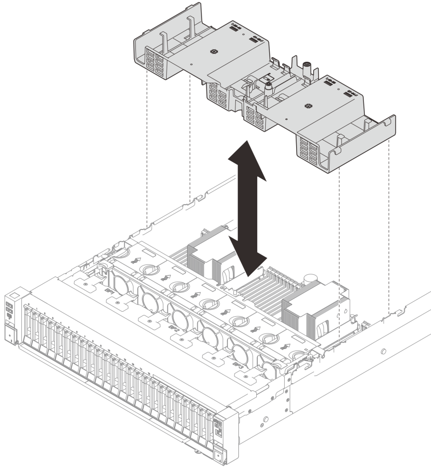
圖例 29. 卸下前方空氣擋板
