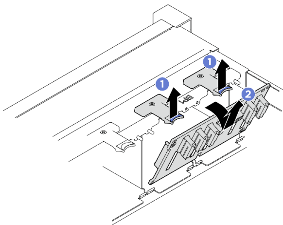
圖例 24. 卸下 2.5 吋硬碟背板
