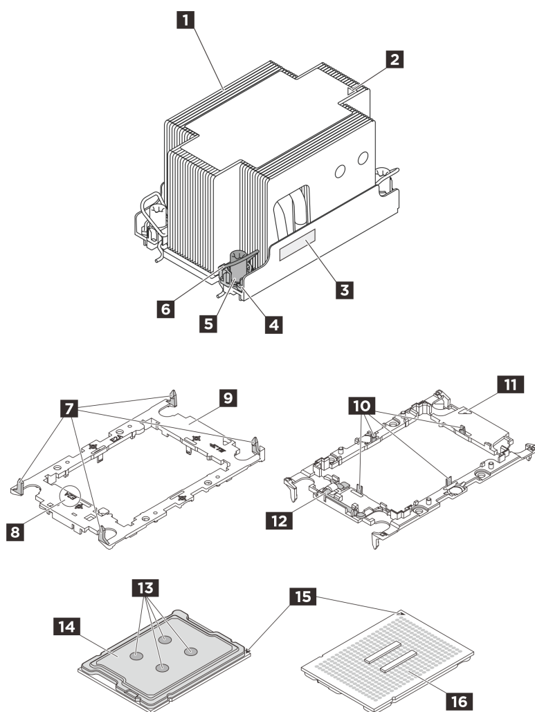
圖例 214. PHM 元件
