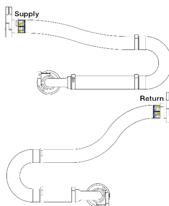
圖例 128. 48U 機架式連接套組
