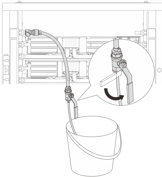
圖例 148. 開啟供應側的洩放閥門
