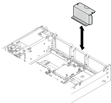
圖例 113. 安裝擴充卡填充板
