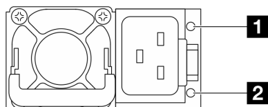
圖例 266. CRPS Premium (CFFv5) 電源供應器上的 LED
