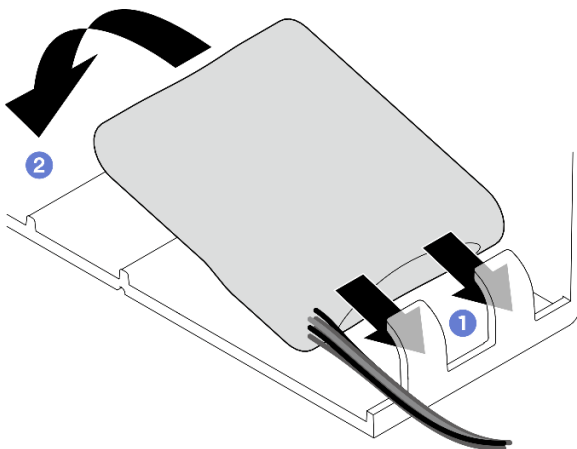
圖例 75. 快閃記憶體電源模組安裝
