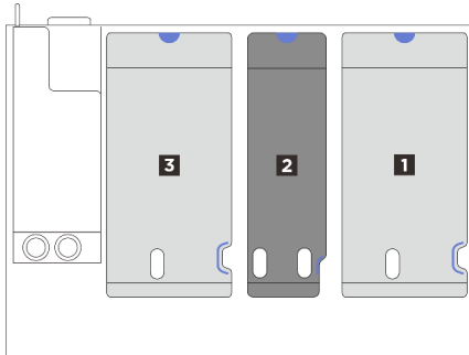
圖例 187. 配備三個 PCIe 擴充卡的伺服器型號
