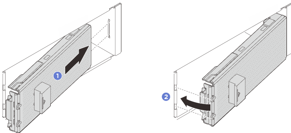
圖例 63. 安裝 E3.S 擋板
