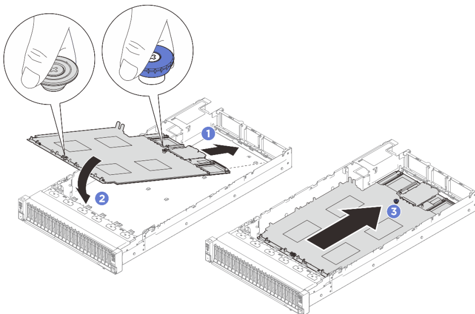
圖例 250. 安裝主機板組件
