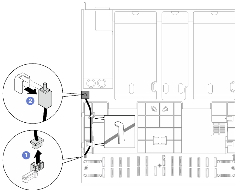
圖例 94. 卸下入侵開關
