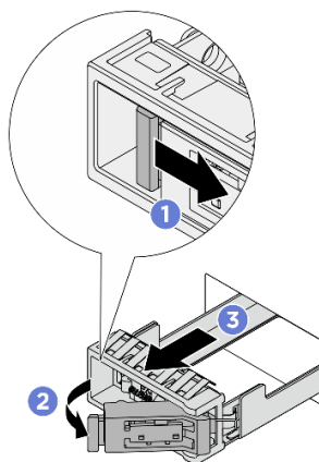
圖例 92. 卸下 M.2 硬碟匣
