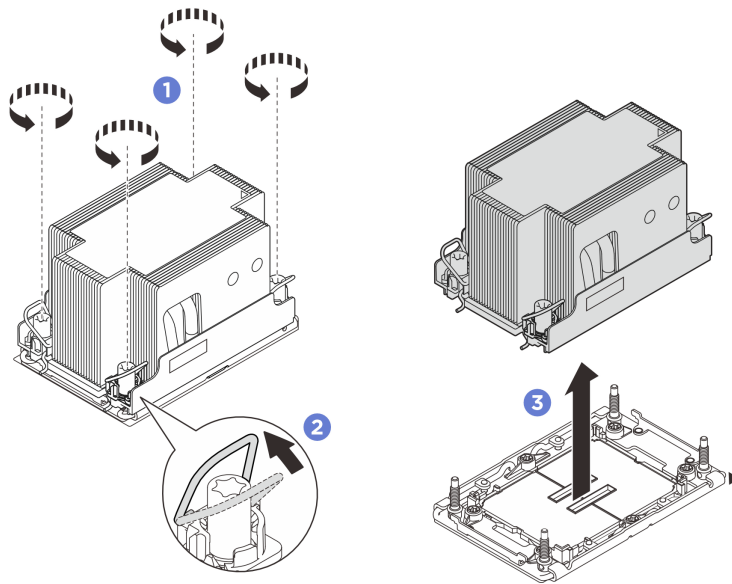
圖例 210. 卸下 2U 標準 PHM
