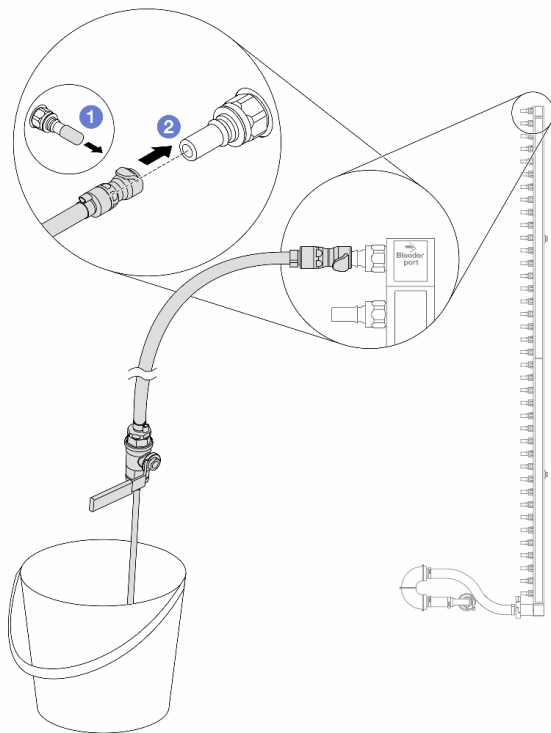
圖例 135. 在回流側安裝洩放套件
