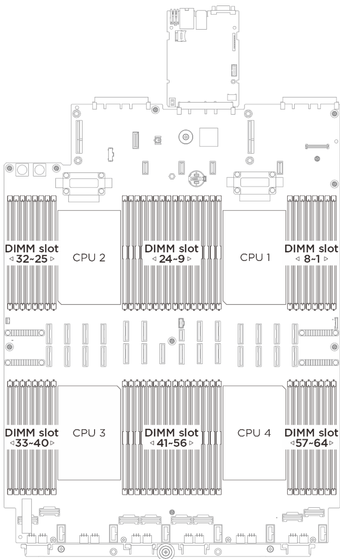
圖例 173. 記憶體模組和處理器佈置
