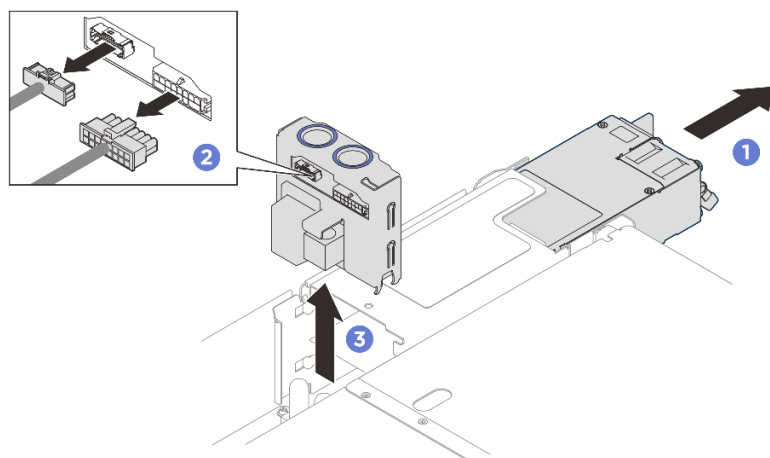
圖例 204. 卸下電源配送板
