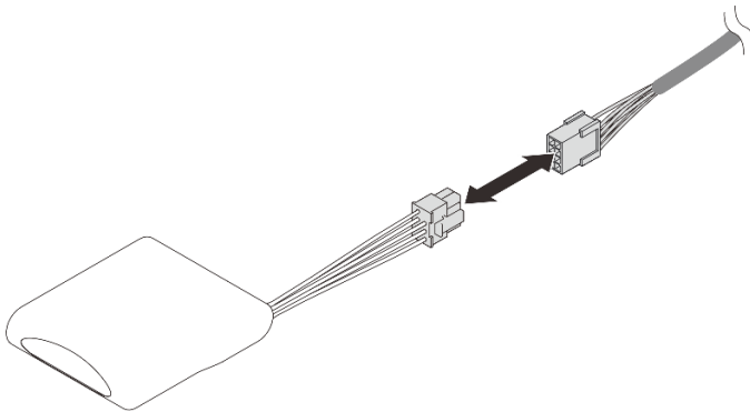
圖例 33. 拔掉快閃記憶體電源模組纜線
