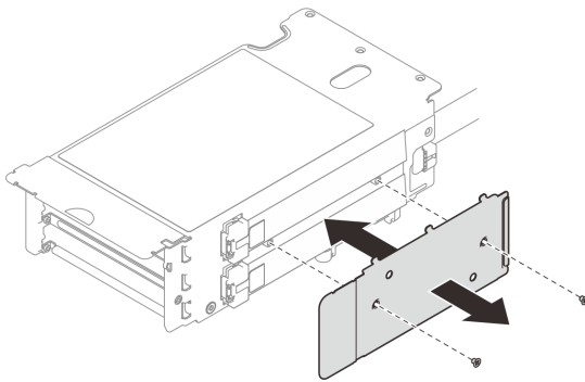
圖例 199. 安裝纜線蓋
