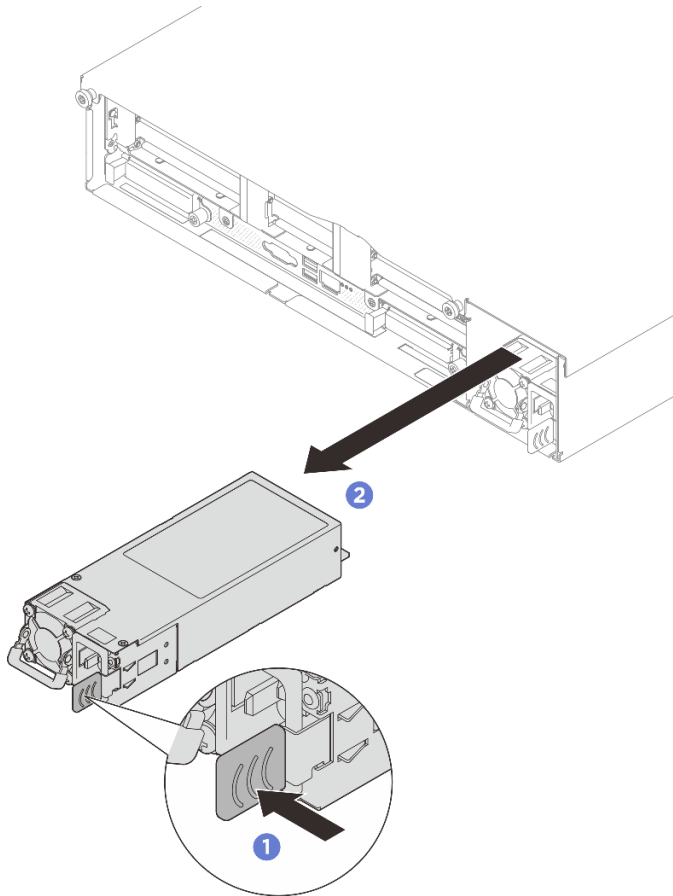
圖例 207. 電源供應器卸下
