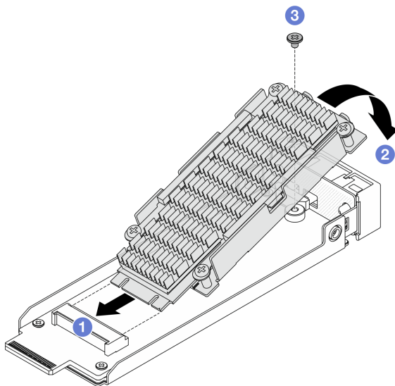
圖例 91. 安裝帶散熱槽的 M.2 硬碟
