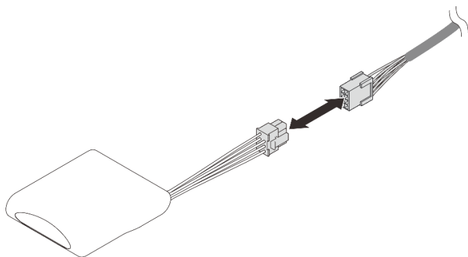
圖例 76. 連接快閃記憶體電源模組纜線
