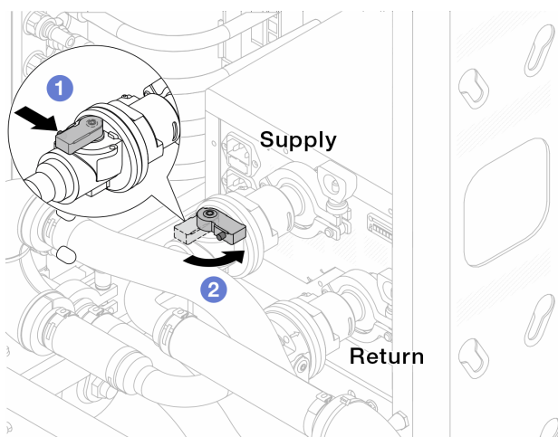
圖例 129. 關閉球閥
