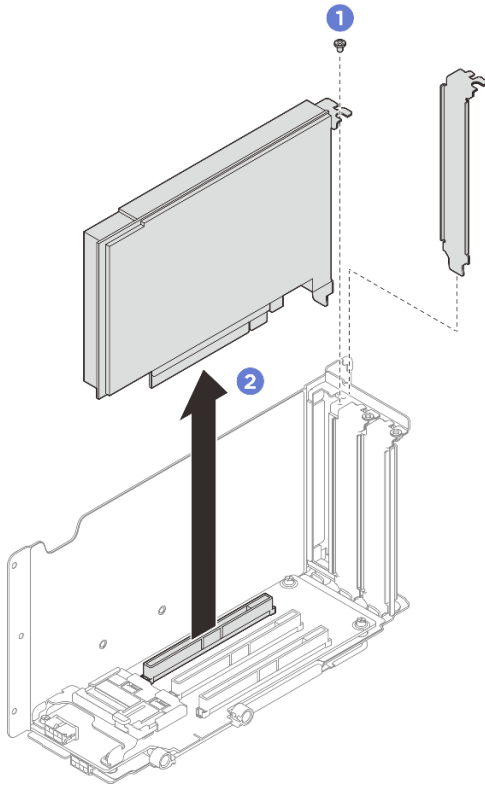
圖例 185. 卸下 PCIe 配接卡
