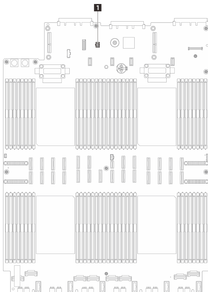
圖例 114. 連接洩漏偵測感應器模組
