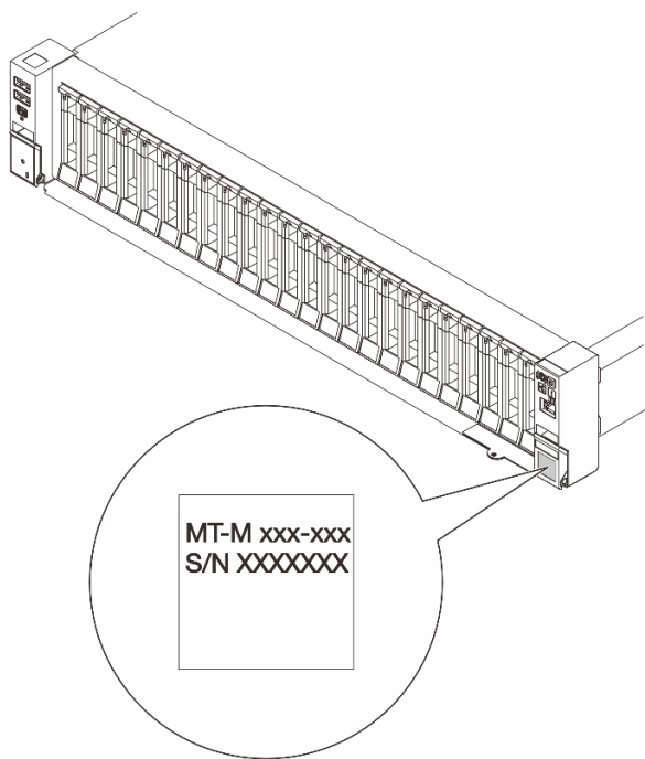
圖例 17. ID 標籤的位置
