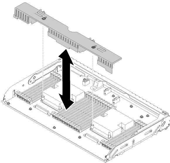
그림 75. 프로세서 및 메모리 확장 트레이에서 공기 조절 장치 제거
