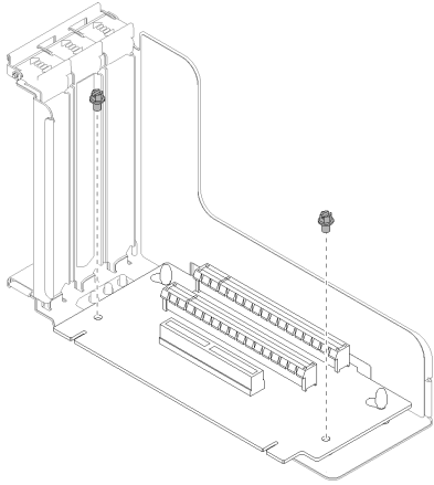
그림 92. PCIe 라이저 카드 어셈블리 분해
