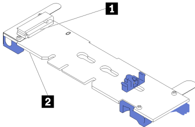
그림 72. M.2 드라이브 슬롯
