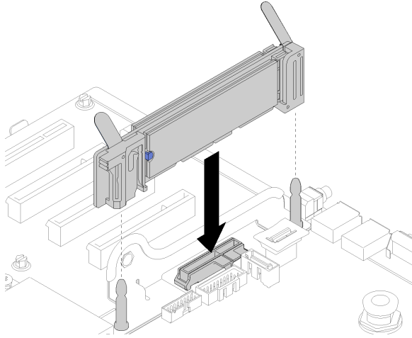
그림 70. M.2 백플레인 설치
