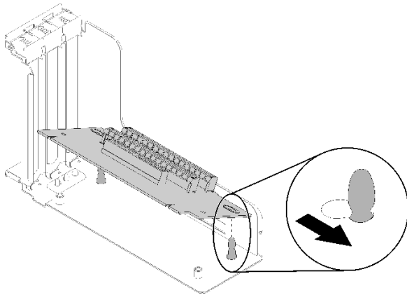
그림 95. PCI 라이저 카드 어셈블리
