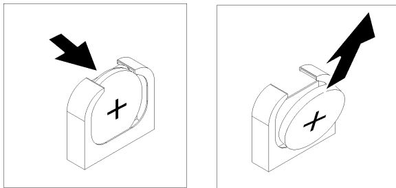
그림 47. CMOS 배터리 제거
