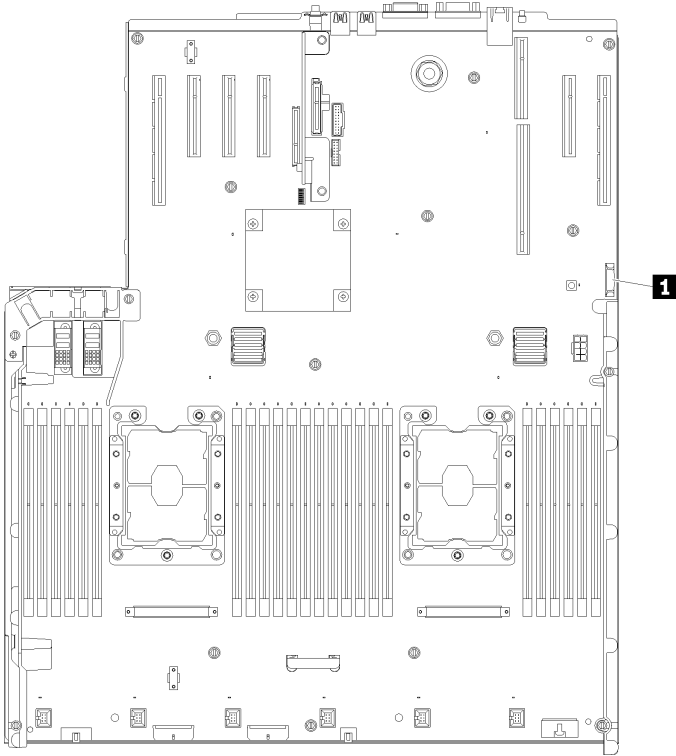
그림 46. 시스템 보드에서 CMOS 배터리 위치
