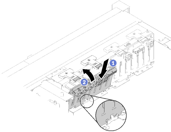
그림 43. 드라이브 백플레인 설치
