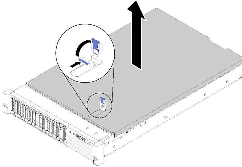
그림 137. 윗면 덮개 제거
