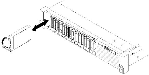
그림 44. 드라이브 제거
