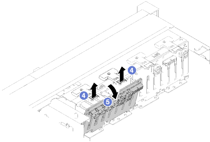
그림 42. 드라이브 백플레인 제거
