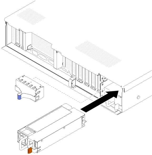
그림 105. 전원 공급 장치 설치
