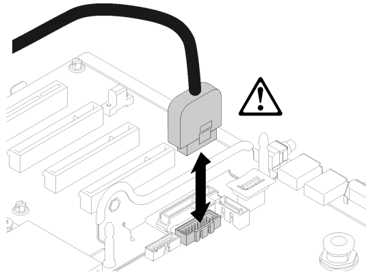
그림 86. USB 3.0 케이블 연결
