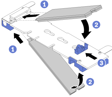
그림 73. M.2 드라이브 설치
