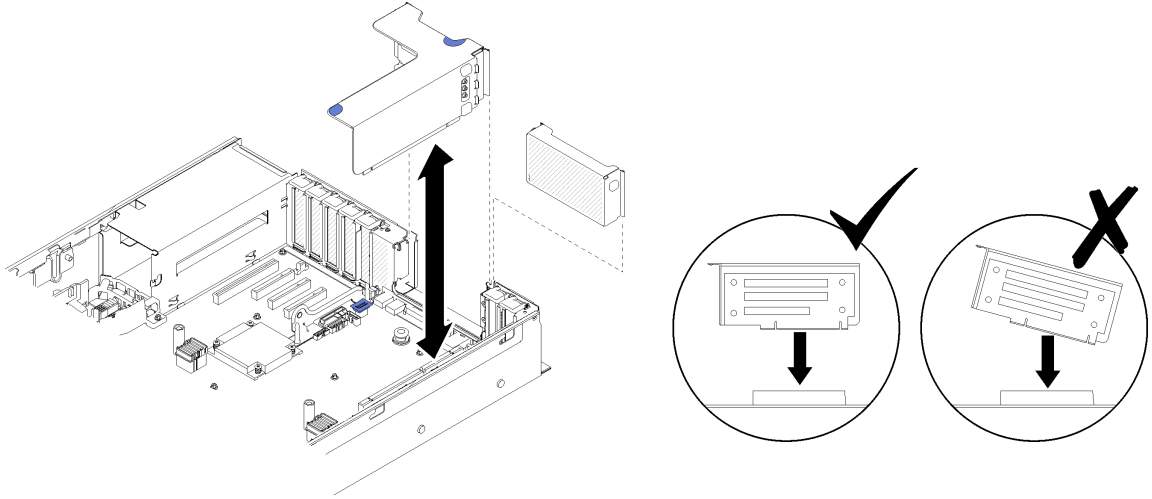
그림 90. PCI 라이저 카드 어셈블리 제거
