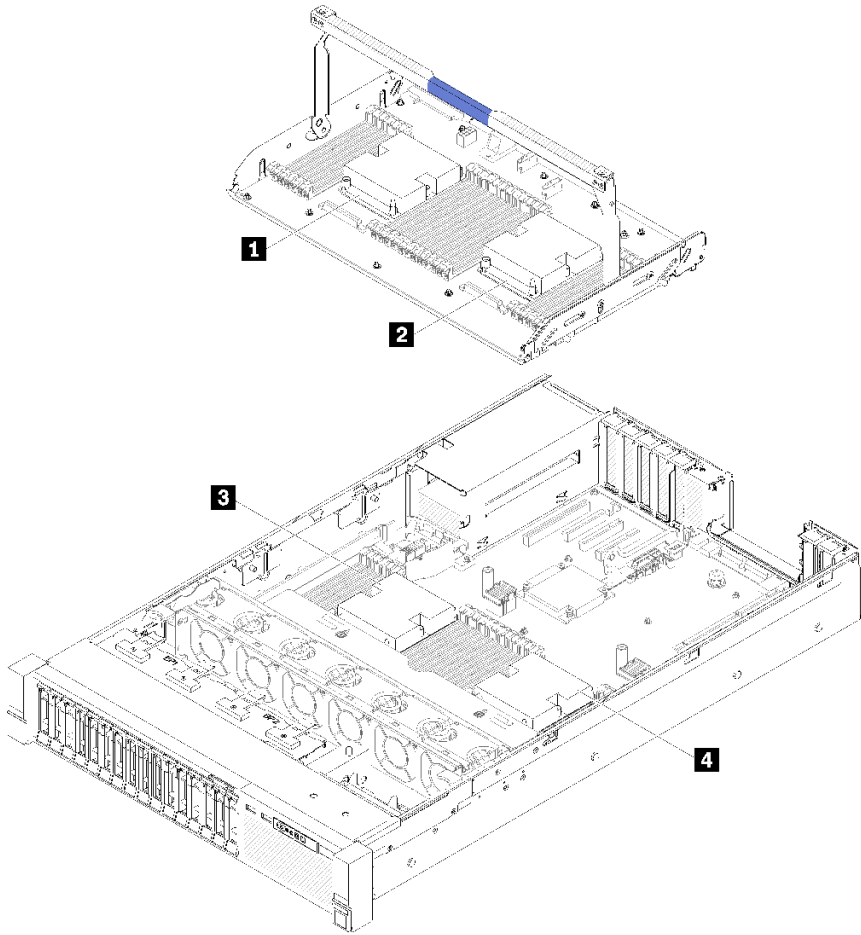
그림 106. 프로세서 위치
