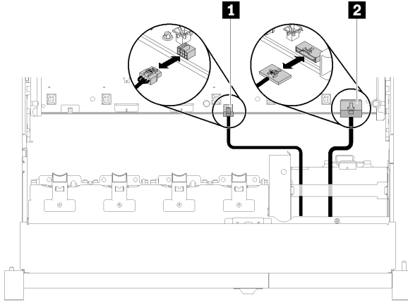
그림 81. USB 2.0 케이블 및 앞면 오퍼레이터 패널 케이블
