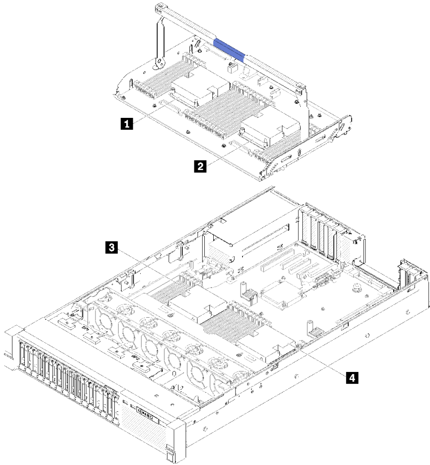
그림 113. 프로세서 위치
