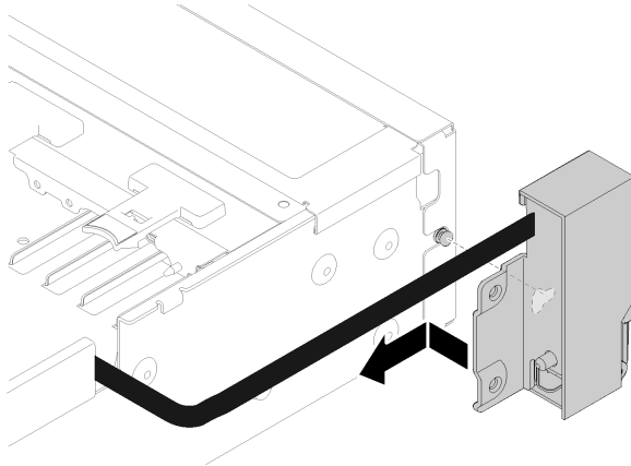
그림 58. 앞면 VGA 어셈블리 설치
