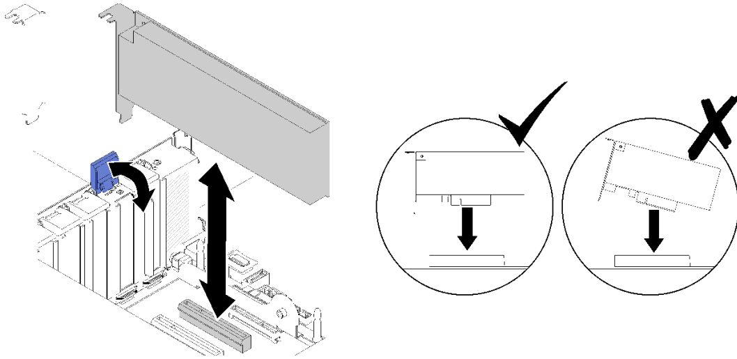
그림 100. 시스템 보드에 어댑터 설치
