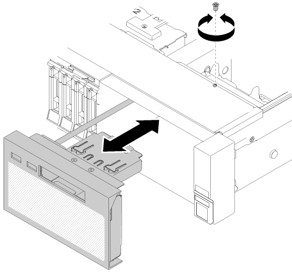
그림 84. 오퍼레이터 패널 트레이 어셈블리 설치
