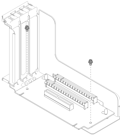
그림 91. PCIe 라이저 카드 제거
