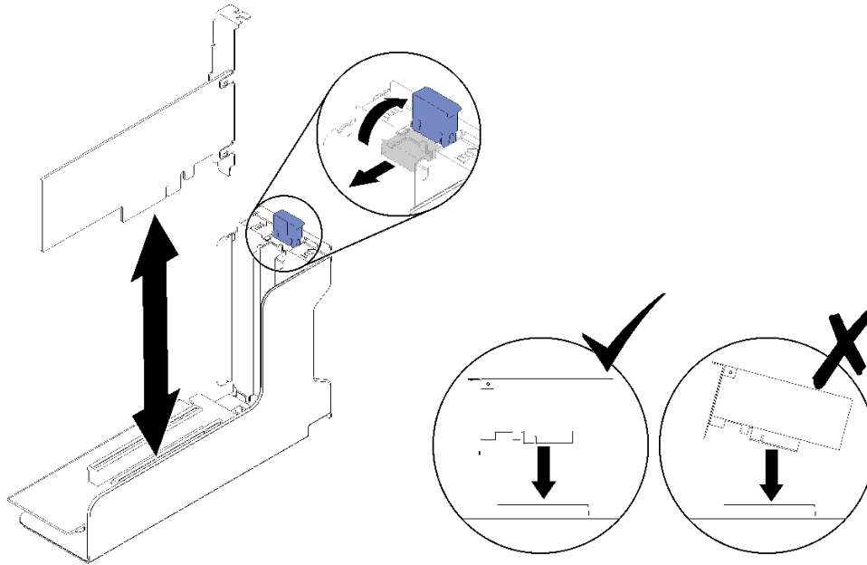
그림 101. PCI 라이저 카드 어셈블리에 어댑터 설치
