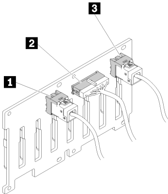
그림 20. 2.5인치 SATA/SAS 8베이 백플레인트
