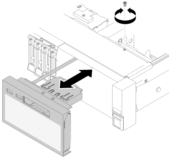
그림 83. 오퍼레이터 패널 트레이 어셈블리 제거
