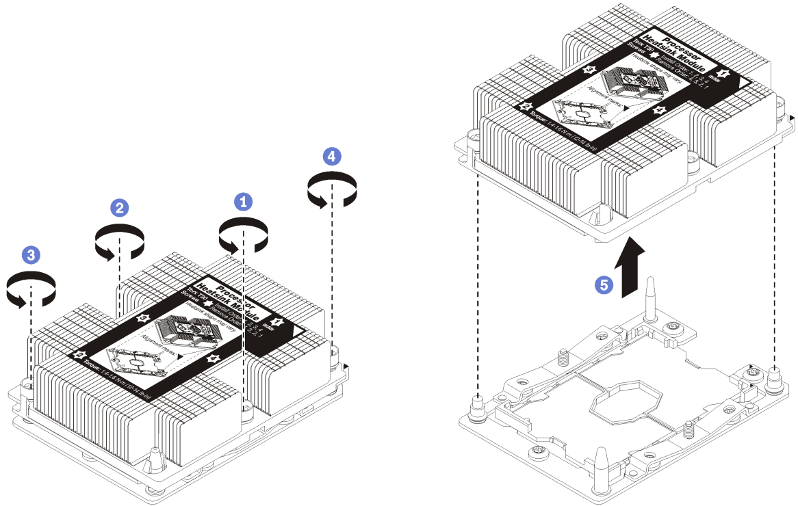
그림 107. PHM 제거
