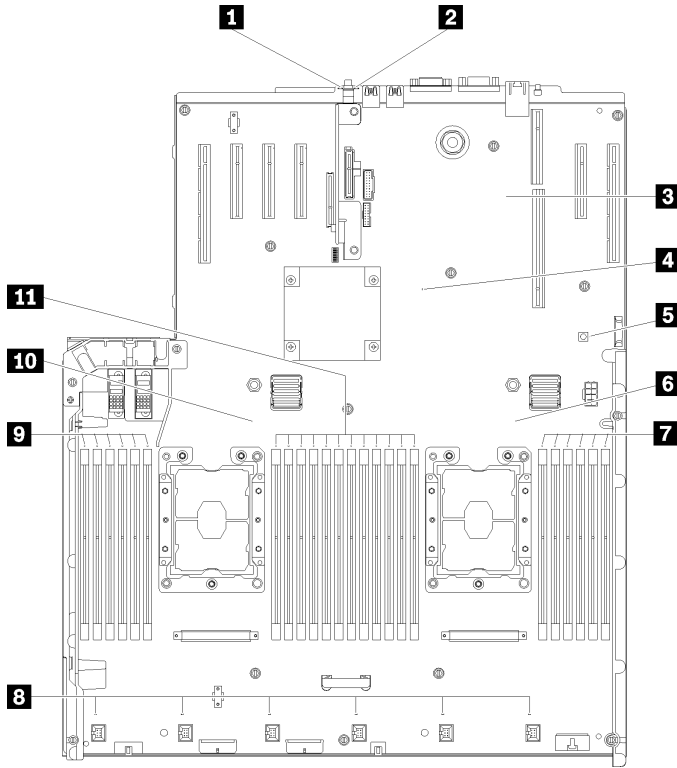
그림 13. 시스템 보드 LED
