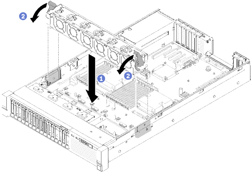
그림 50. 팬 케이스 어셈블리 설치
