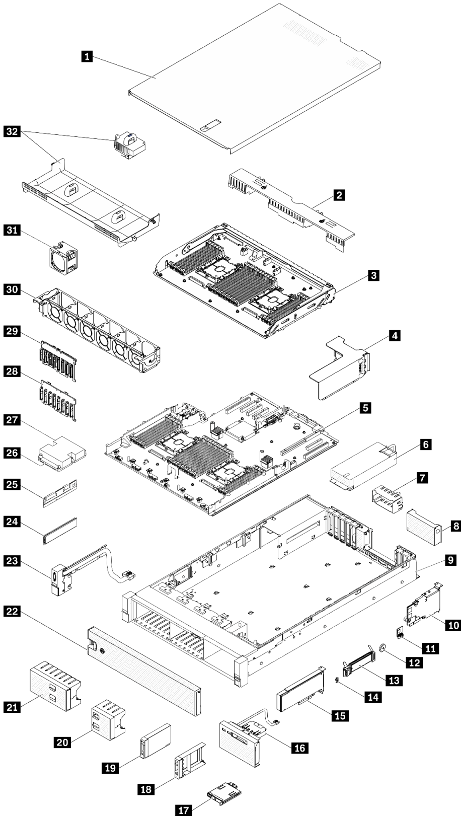
그림 41. 서버 구성 요소
