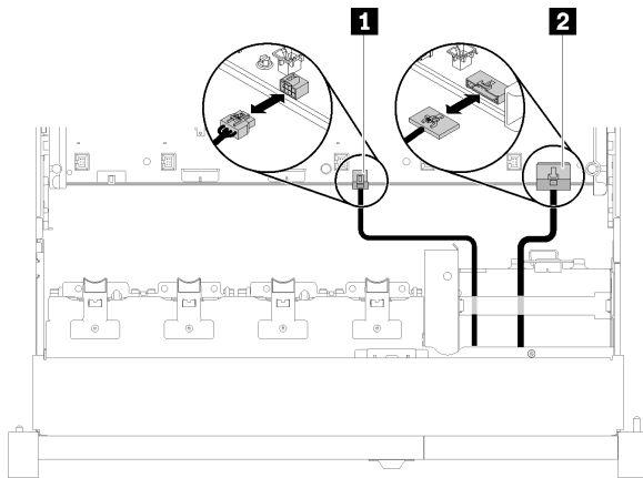
그림 85. USB 2.0 케이블 및 앞면 오퍼레이터 패널 케이블
