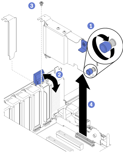
그림 62. LOM 어댑터 제거
