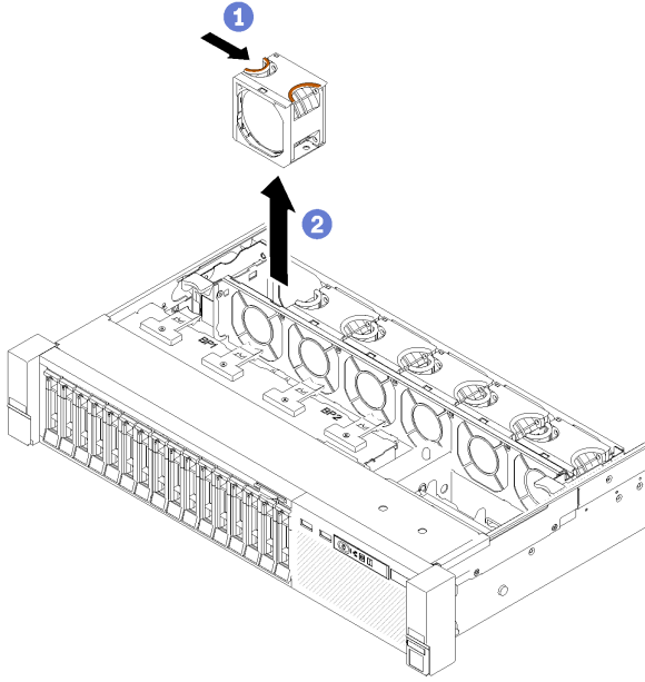
그림 51. 핫 스왑 팬 제거
