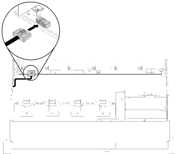
그림 61. 앞면 VGA 어셈블리 설치
