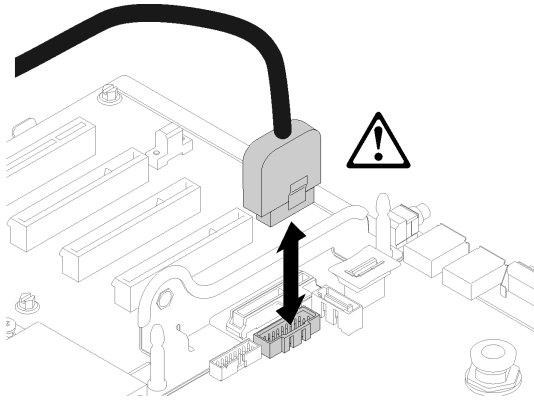
그림 134. USB 3.0 커넥터를 수직으로 제거
