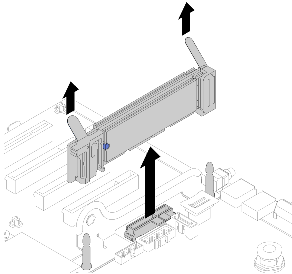
그림 68. M.2 백플레인 제거
