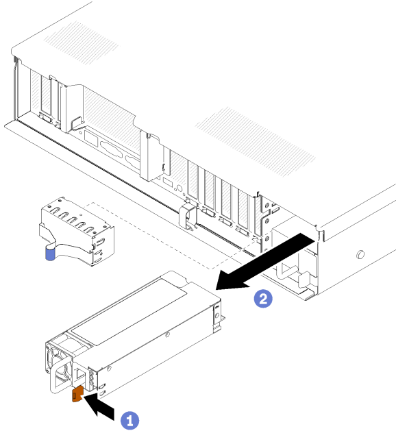
그림 103. 전원 공급 장치 유닛 제거
