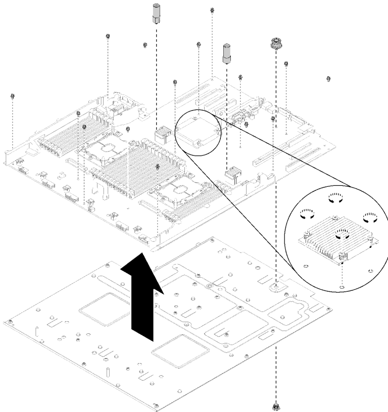
그림 143. 시스템 보드 분해
