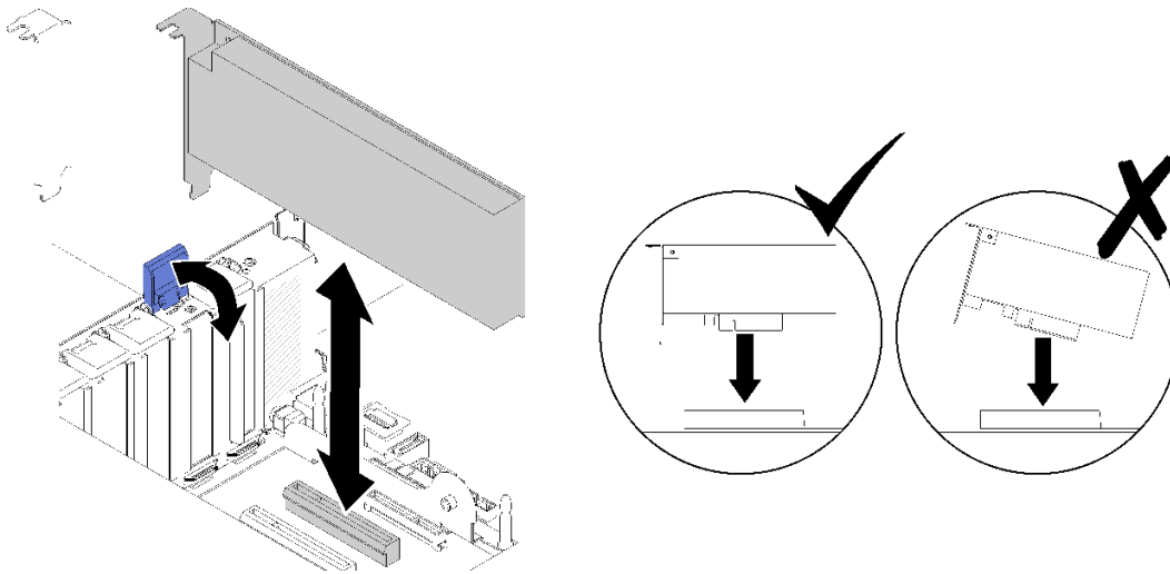
그림 98. 시스템 보드에서 어댑터 제거
