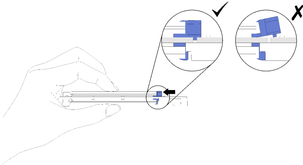
그림 74. 고정장치를 사용해서 M.2 드라이브를 제자리에 설치
