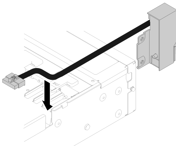
그림 57. 앞면 VGA 어셈블리 설치
