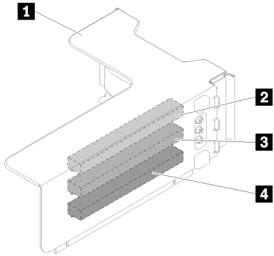
그림 17. x8/x8/x8 PCIe FH 라이저 어셈블리
