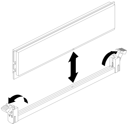
그림 77. 메모리 모듈 제거
