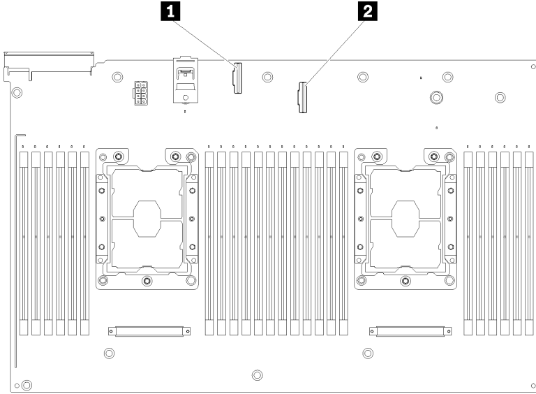
그림 16. 옵션 프로세서 및 메모리 확장 트레이의 커넥터
