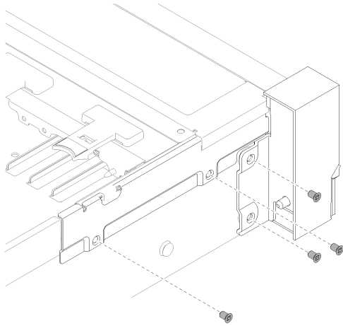
그림 54. 앞면 VGA 어셈블리 제거
