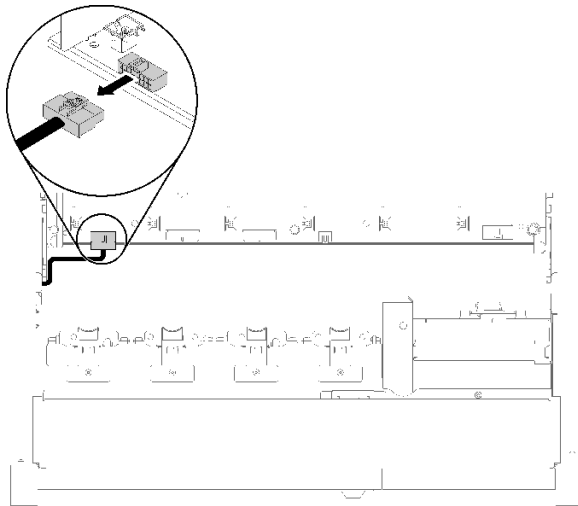
그림 53. 시스템 보드에서 앞면 VGA 커넥터의 위치
