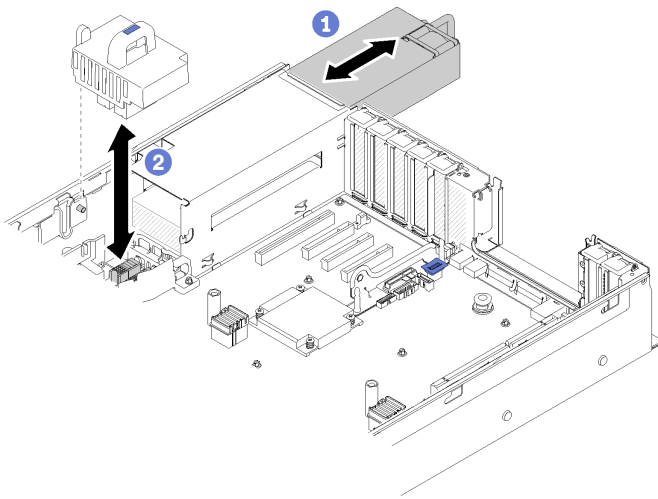
그림 124. 전원 인터포저 제거
