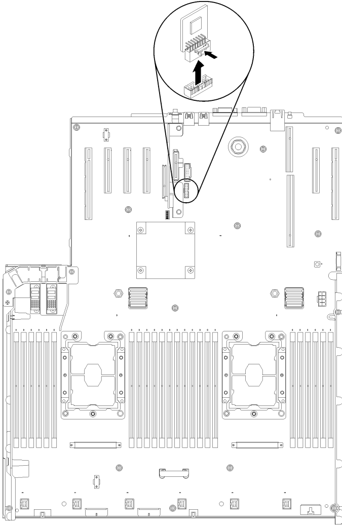
그림 133. TCM/TPM 어댑터 제거
