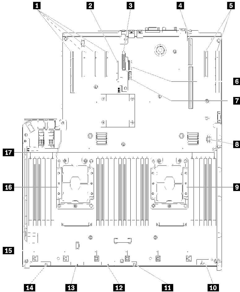
그림 11. 시스템 보드 커넥터
