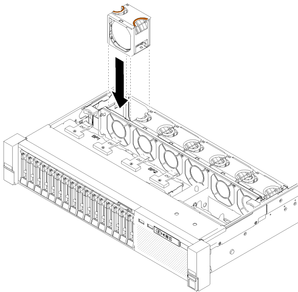
그림 52. 핫 스왑 팬 설치
