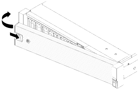
그림 121. 보안 베젤 제거
