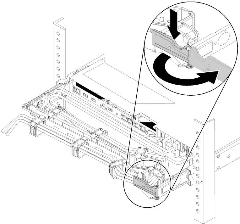
그림 102. CMA 조정
