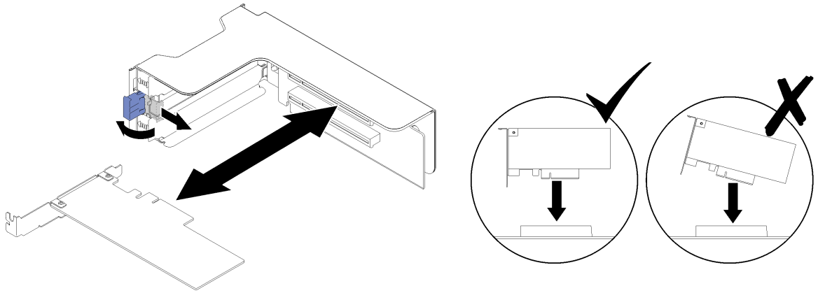
그림 99. PCI 라이저 카드 어셈블리에서 어댑터 제거
