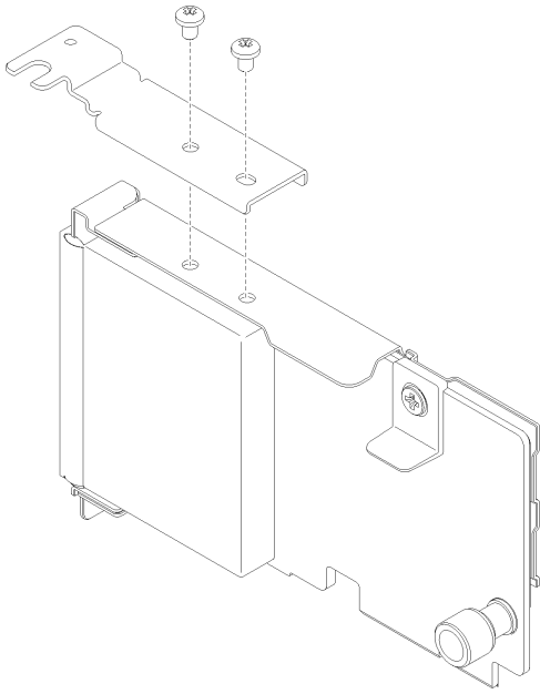
그림 64. LOM 어댑터 어셈블리
