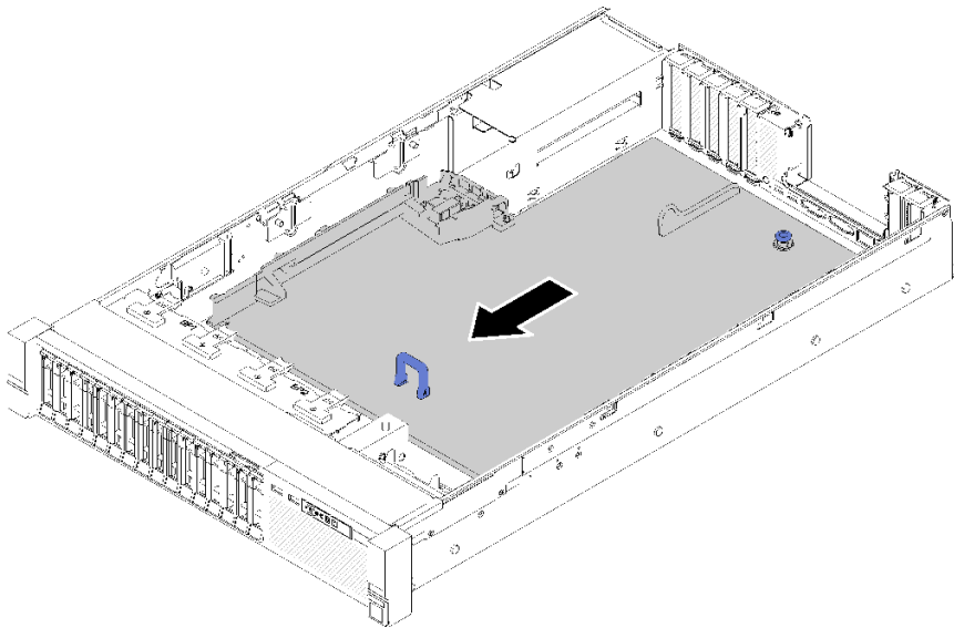
그림 129. 시스템 보드 제거
