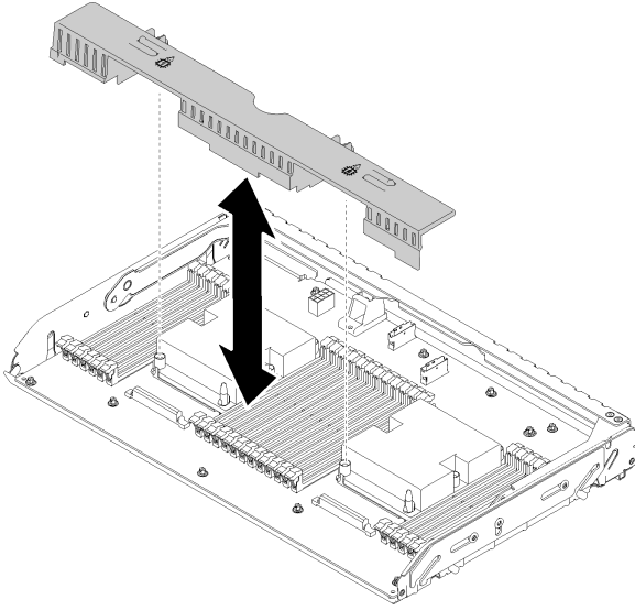
그림 119. 확장 트레이 공기 조절 장치 설치
