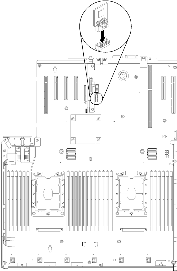
그림 135. TCM/TPM 어댑터 설치
