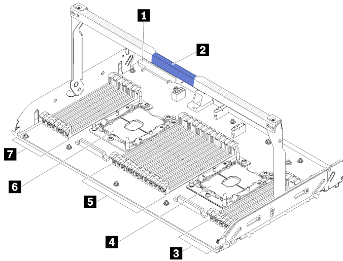
그림 14. 옵션 프로세서 및 메모리 확장 트레이
