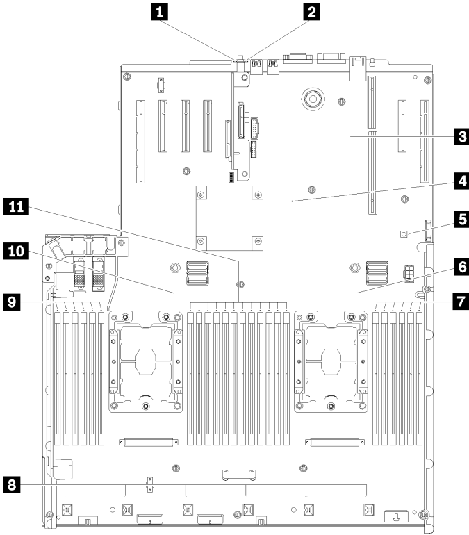
그림 142. 시스템 보드 LED
