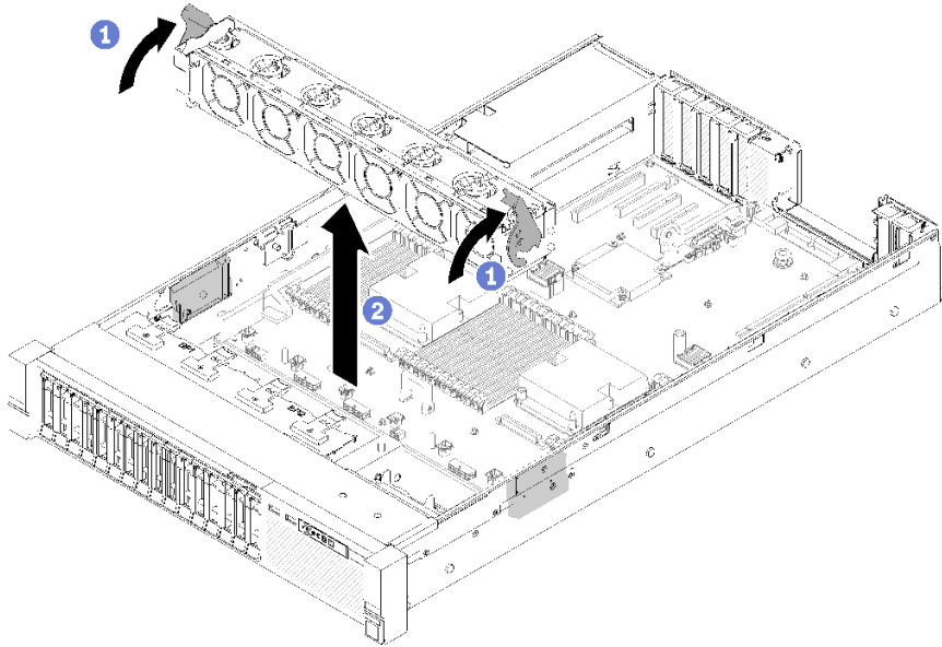
그림 49. 팬 케이스 어셈블리 제거
