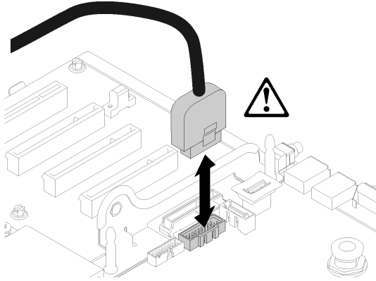
그림 132. USB 3.0 커넥터를 수직으로 제거
