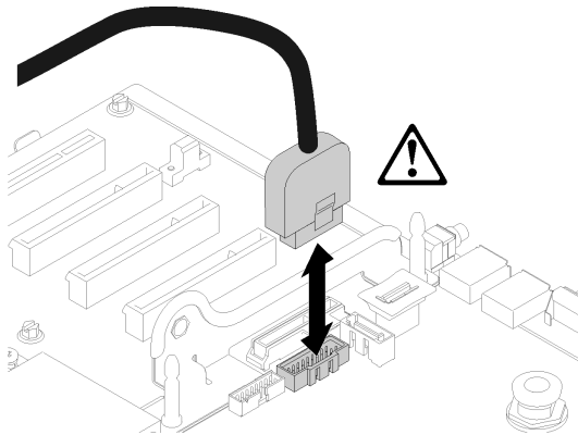
그림 82. USB 3.0 커넥터를 수직으로 제거
