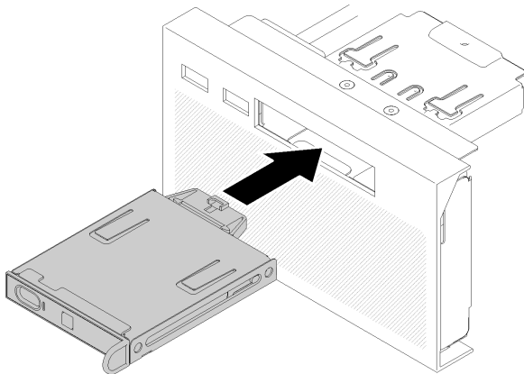
그림 88. 앞면 오퍼레이터 패널 설치
