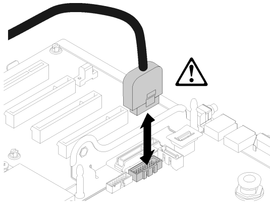
그림 69. USB 3.0 커넥터를 수직으로 제거
