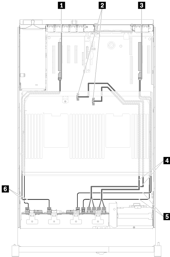
그림 36. 케이블 배선, 8베이 백플레인 + AnyBay 백플레인
