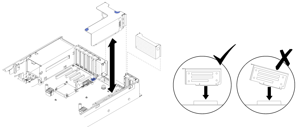
그림 97. PCI 라이저 카드 어셈블리 설치
