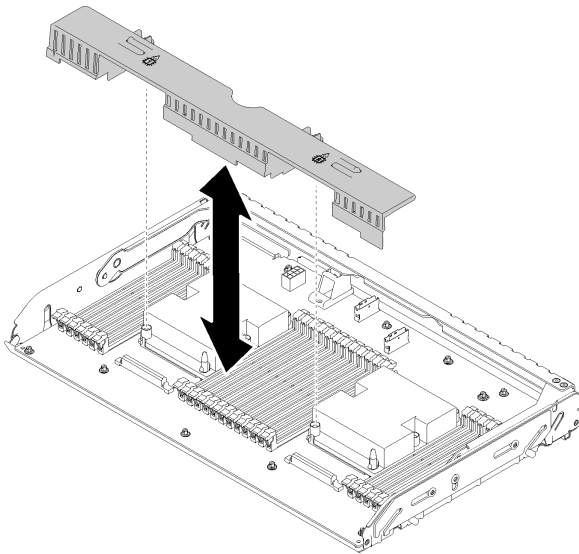
그림 115. 확장 트레이 공기 조절 장치 제거
