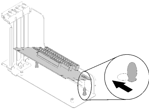
그림 93. PCIe 라이저 카드 어셈블리 분해
