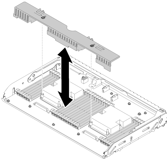
그림 78. 프로세서 및 메모리 확장 트레이에서 공기 조절 장치 제거
