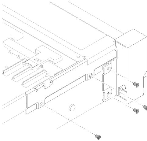
그림 60. 앞면 VGA 어셈블리 설치
