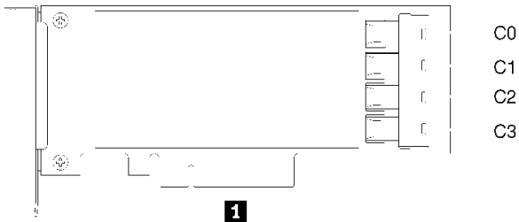
그림 23. SATA/SAS RAID 어댑터(16i)의 커넥터
