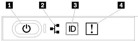
그림 141. 앞면 오퍼레이터 패널
