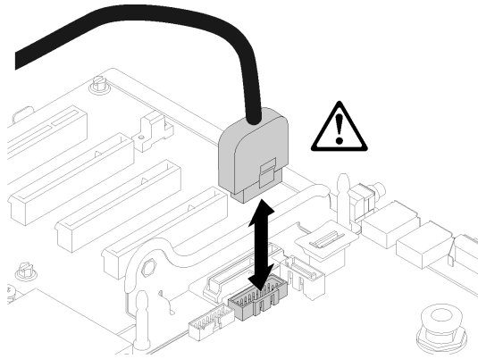
그림 128. USB 3.0을 수직으로 분리
