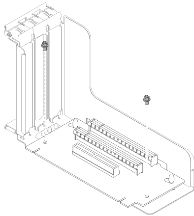
그림 96. PCI 라이저 카드 어셈블리
