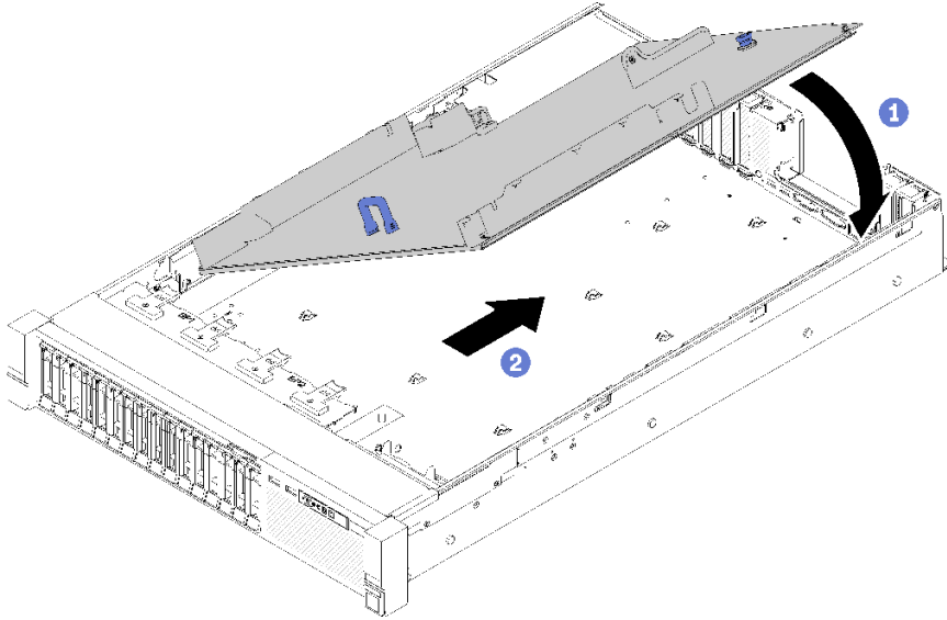
그림 131. 시스템 보드 설치
