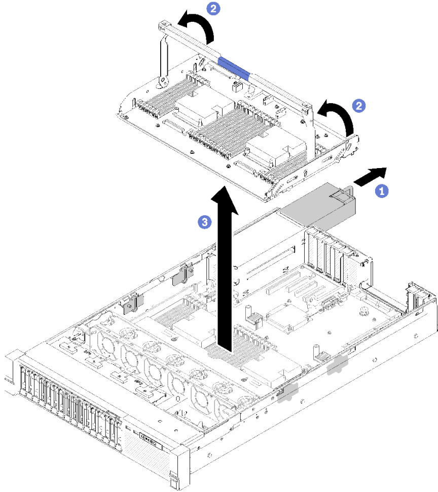
그림 116. 프로세서 및 메모리 확장 트레이 제거
