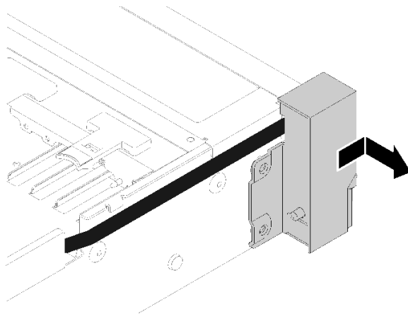
그림 56. 앞면 VGA 어셈블리 제거
