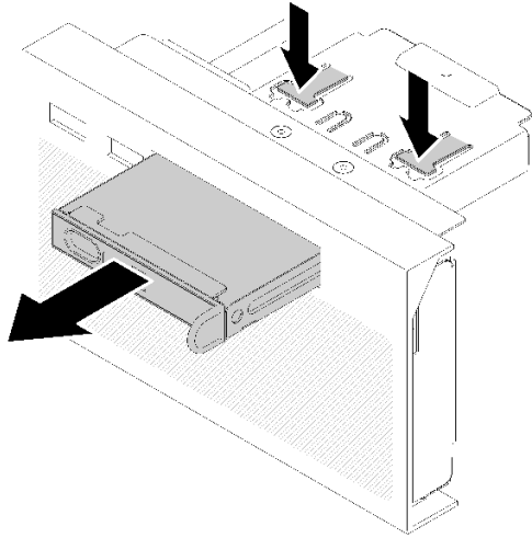
그림 87. 앞면 오퍼레이터 패널 제거
