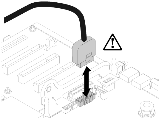
그림 89. USB 3.0 커넥터를 수직으로 제거
