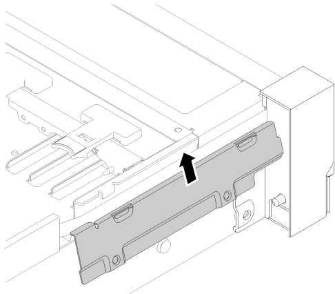
그림 55. 앞면 VGA 어셈블리 제거
