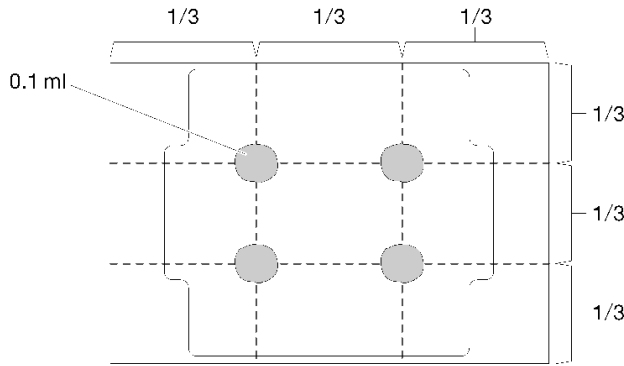
그림 111. 열 그리스의 적절한 형태
