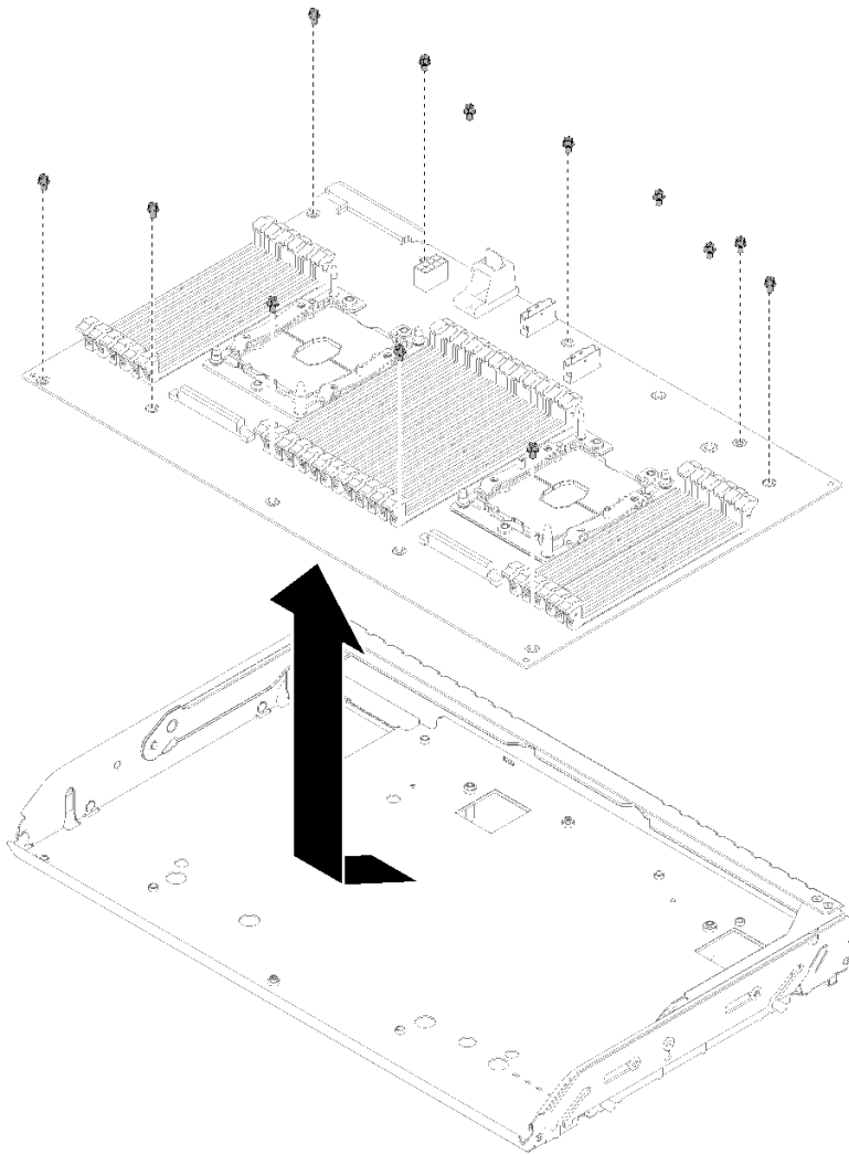
그림 144. 확장 트레이 분해
