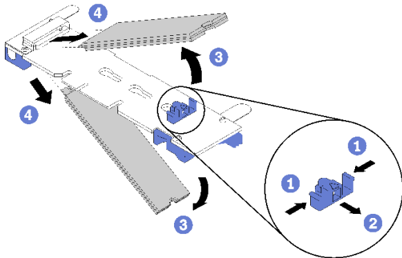
그림 71. M.2 드라이브 제거
