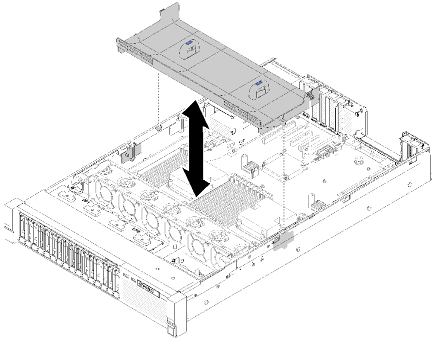
그림 125. 시스템 보드 공기 조절 장치 제거
