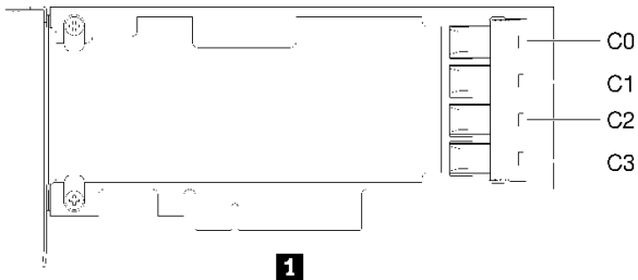
그림 24. PCIe 스위치 카드의 커넥터
