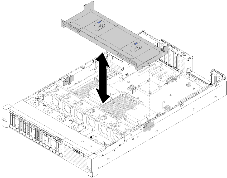
그림 127. 시스템 보드 공기 조절 장치 설치
