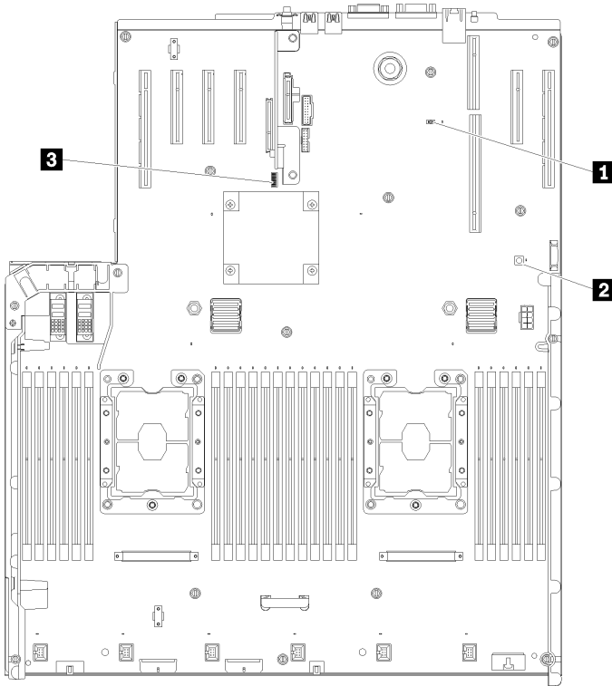
그림 12. 스위치, 점퍼, 버튼
