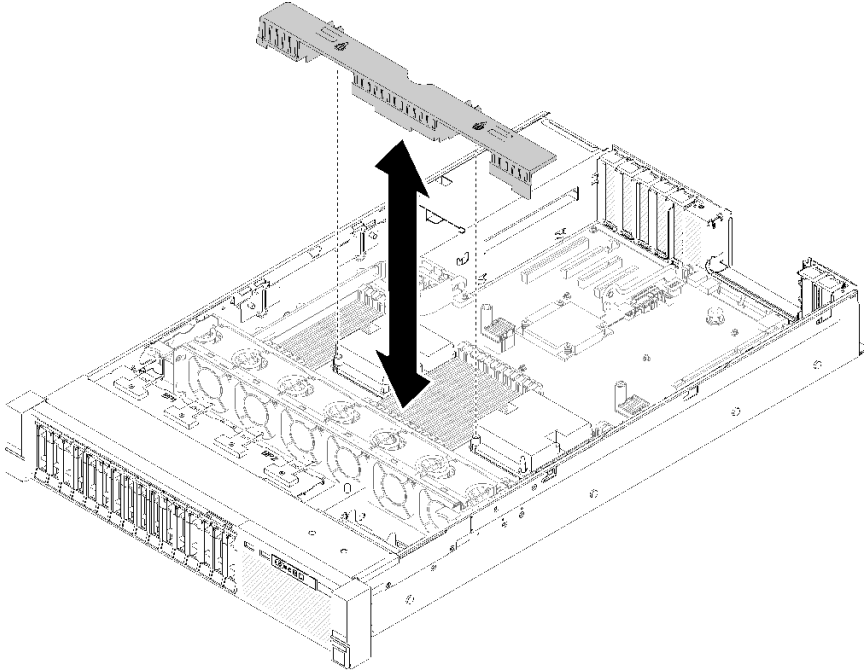
그림 79. 시스템 보드에서 공기 조절 장치 제거
