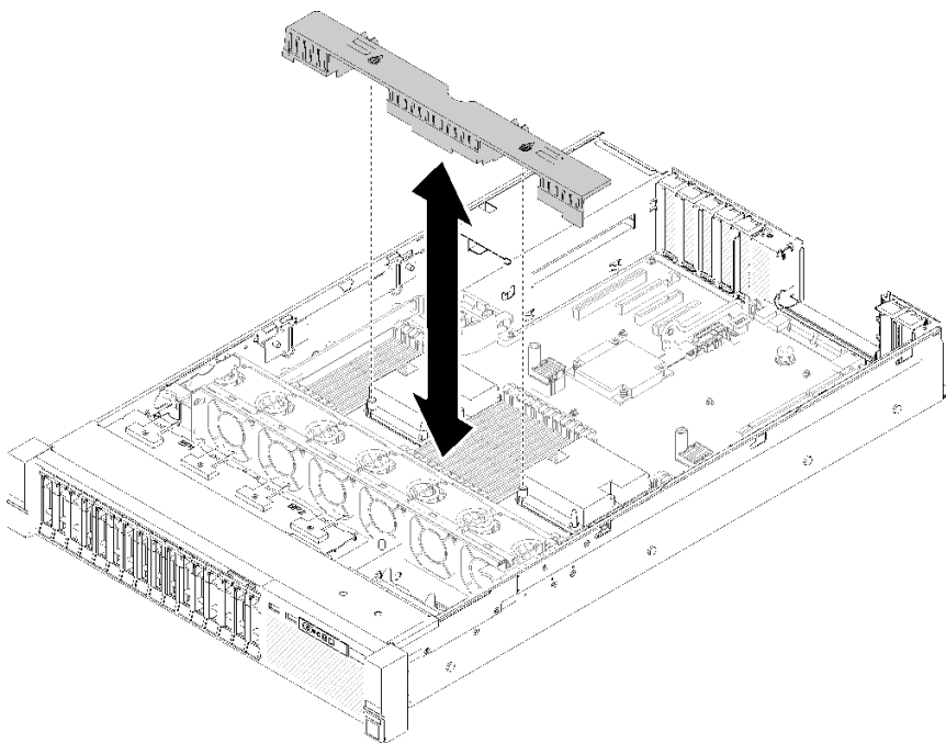
그림 117. 확장 트레이 공기 조절 장치 설치
