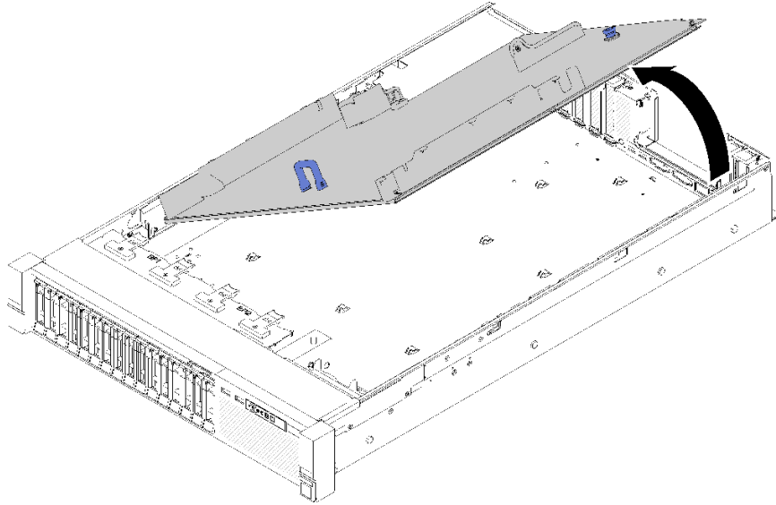
그림 130. 시스템 보드 제거
