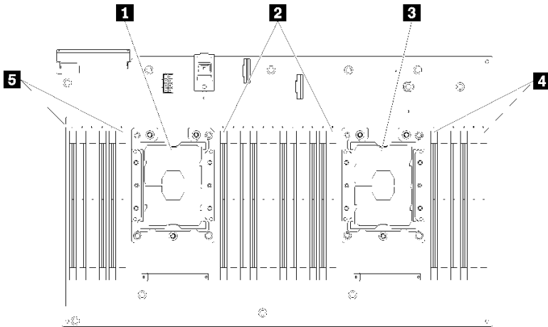
그림 4. 프로세서 및 메모리 모듈 레이아웃: 프로세서 3 및 4
