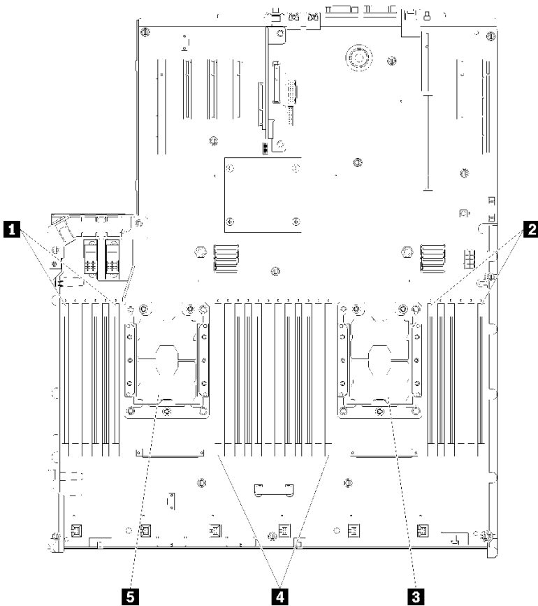
그림 5. 프로세서 및 메모리 모듈 레이아웃: 프로세서 1 및 2
