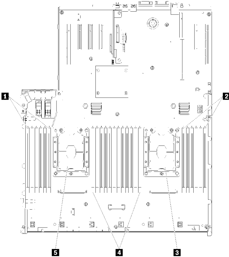
그림 1. 프로세서 및 메모리 모듈 레이아웃: 프로세서 1 및 2
