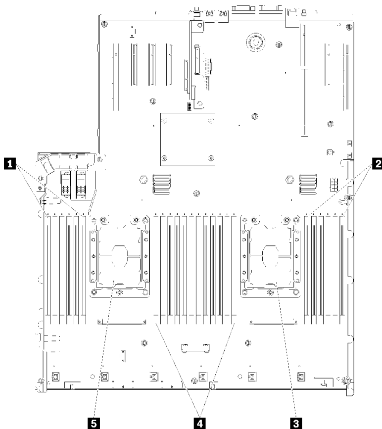
그림 3. 프로세서 및 메모리 모듈 레이아웃: 프로세서 1 및 2
