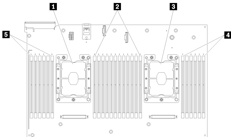
图 4. 处理器和内存条布局: 处理器 3 和 4
