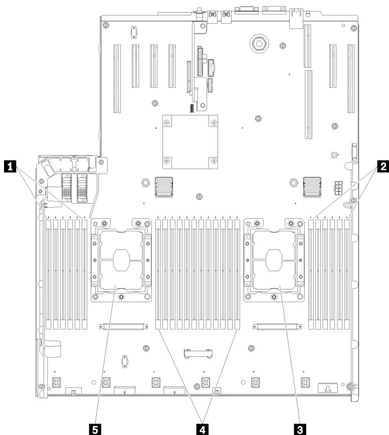
图 3. 处理器和内存条布局：处理器 1 和 2
