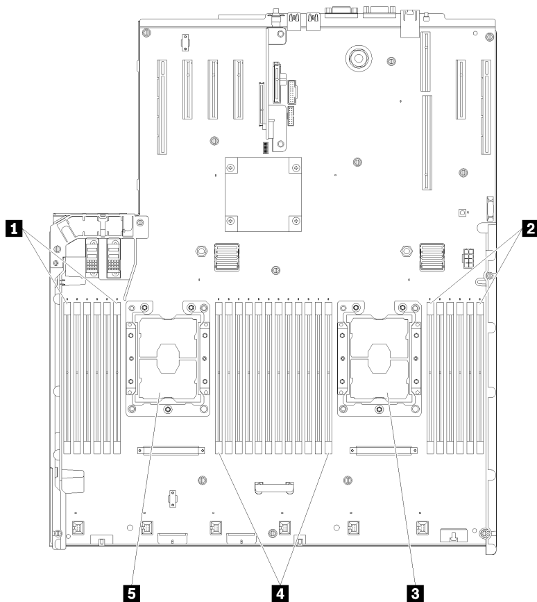
图 5. 处理器和内存条布局：处理器 1 和 2
