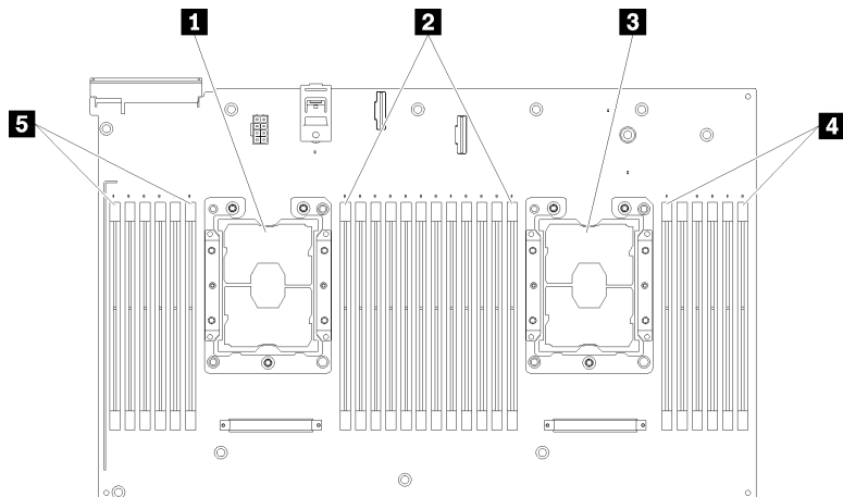
图 2. 处理器和内存条布局：处理器 3 和 4
