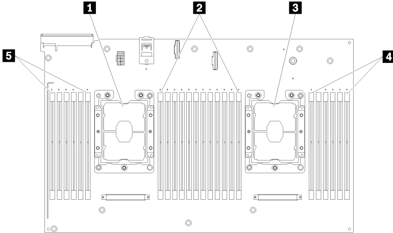
图 6. 处理器和内存条布局：处理器 3 和 4
