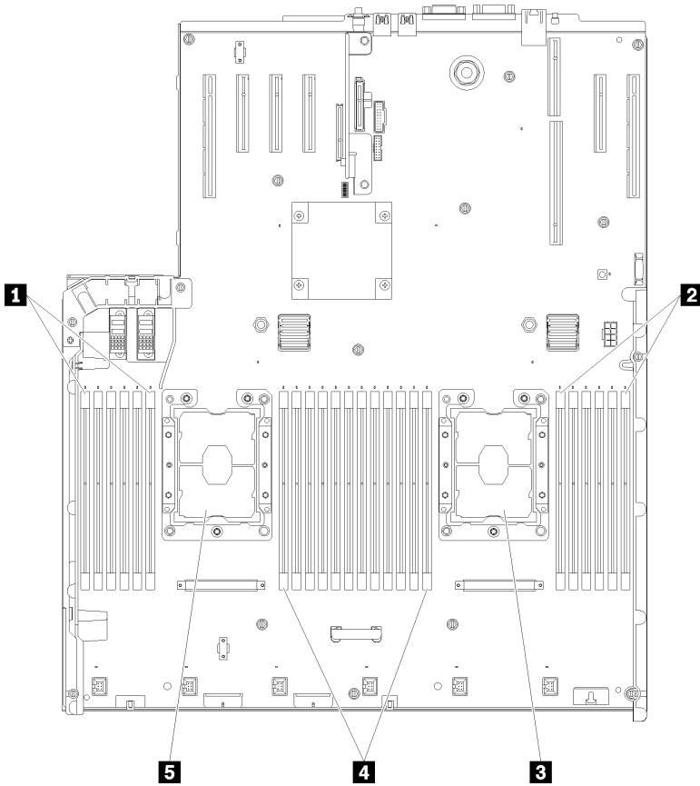
图 1. 处理器和内存条布局：处理器 1 和 2
