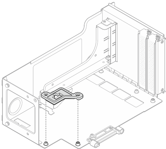
Figura 137. Instalación de la guía del conector a la expansión
