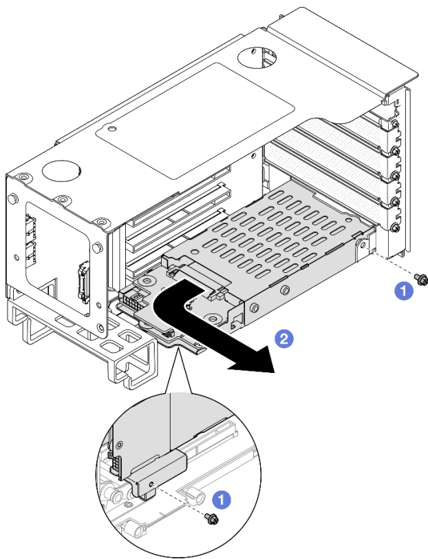
Figura 9. Extracción del compartimiento de la unidad de 7 mm de la expansión
