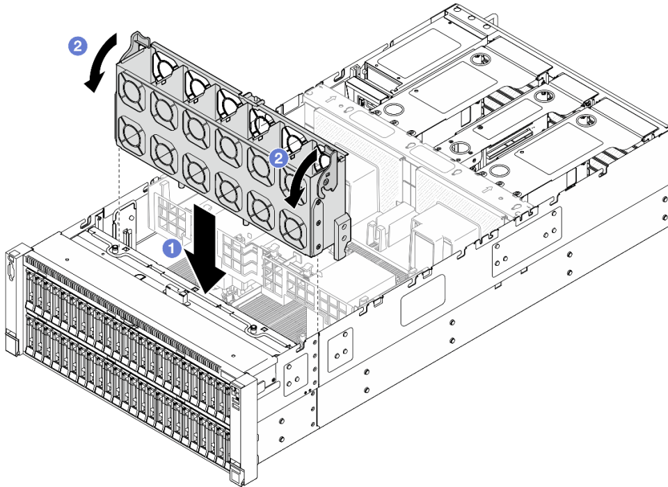
Figura 66. Instalación del compartimiento del ventilador
