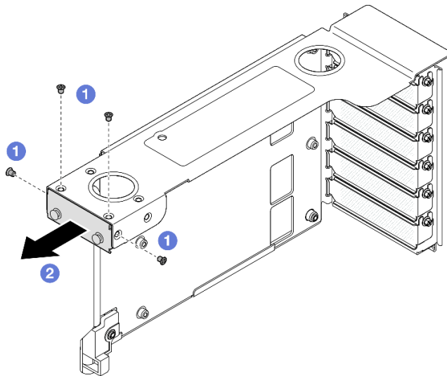
Figura 160. Extracción del relleno de la expansión FH de PCIe
