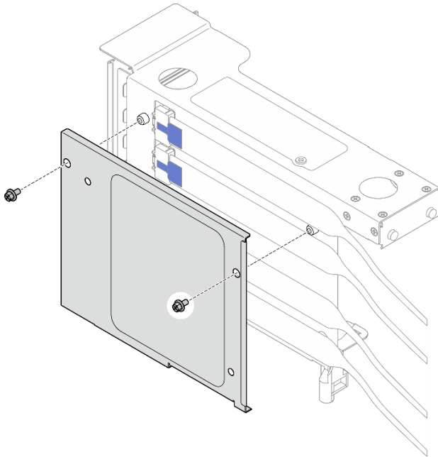
Figura 132. Extracción de la cubierta de la expansión
