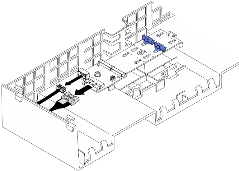
Figura 23. Desconexión del cable del adaptador de arranque M.2 SATA/x4 NVMe
