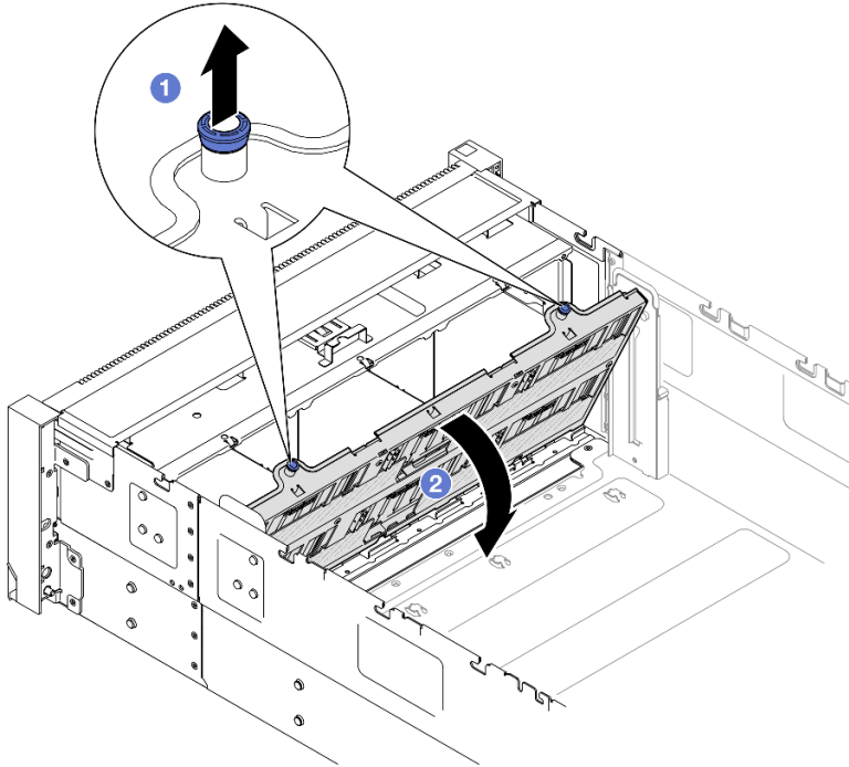
Figura 57. Extracción del conjunto del transportador de la placa posterior de unidad
