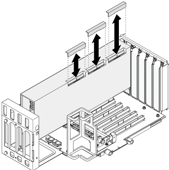
Figura 73. Instalación de la cubierta del conector de enlace en la GPU
