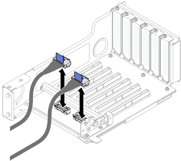
Figura 152. Conexión de los cables de la expansión de PCIe al interior de la expansión
