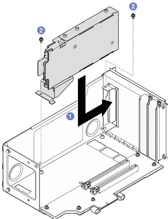
Figura 16. Instalación del compartimiento de la unidad de 7 mm en la expansión
