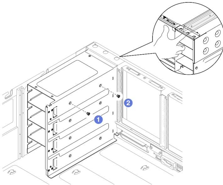
Figura 167. Extracción de tornillo de soporte de fuente de alimentación
