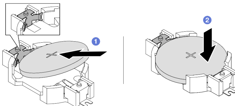
Figura 48. Instalación de la batería CMOS
