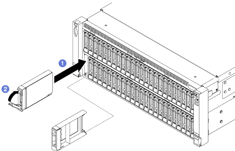
Figura 56. Instalación de una unidad de 2,5 pulgadas
