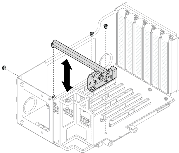
Figura 143. Instalación del elemento de sujeción de PCIe en la expansión
