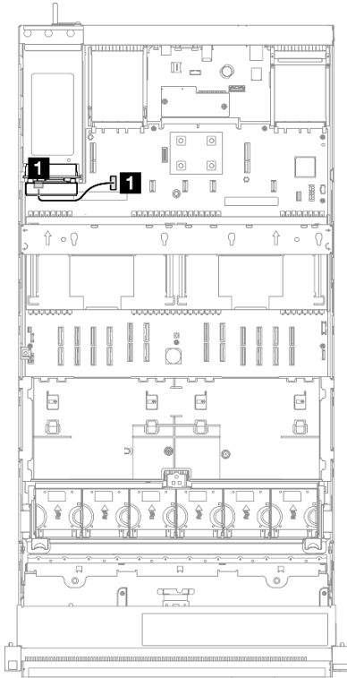
Figura 220. Disposición de los cables de banda lateral para la placa de la distribución de alimentación
