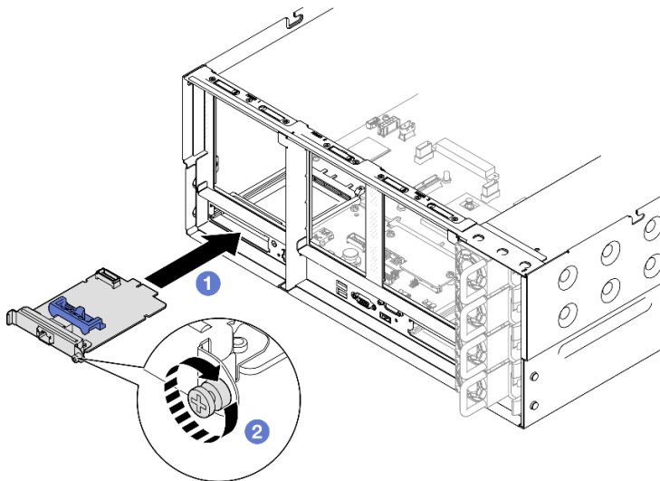
Figura 99. Instalación del adaptador NIC de gestión
