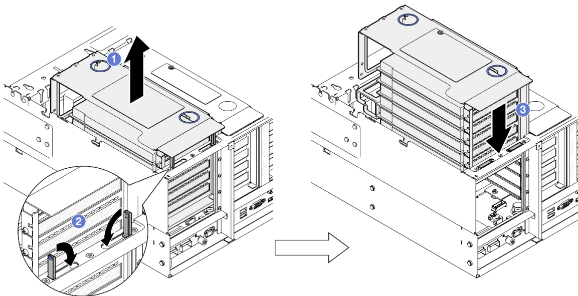
Figura 54. Fijación de la expansión de PCIe
