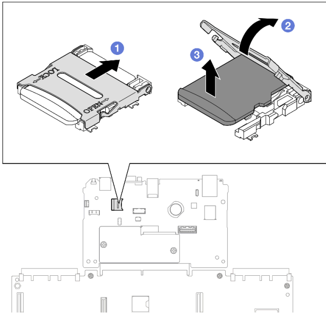
Figura 102. Extraer la tarjeta MicroSD
