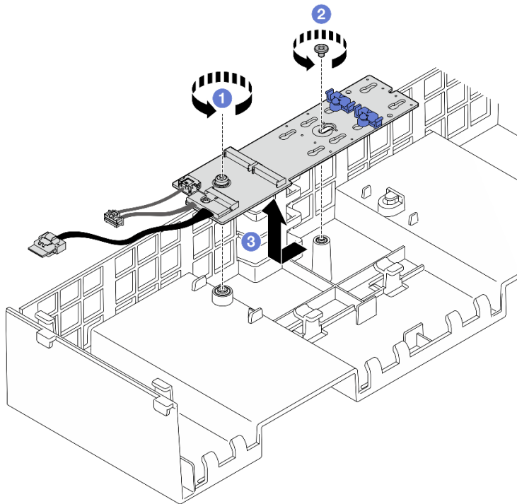
Figura 89. Extracción del adaptador de arranque M.2
