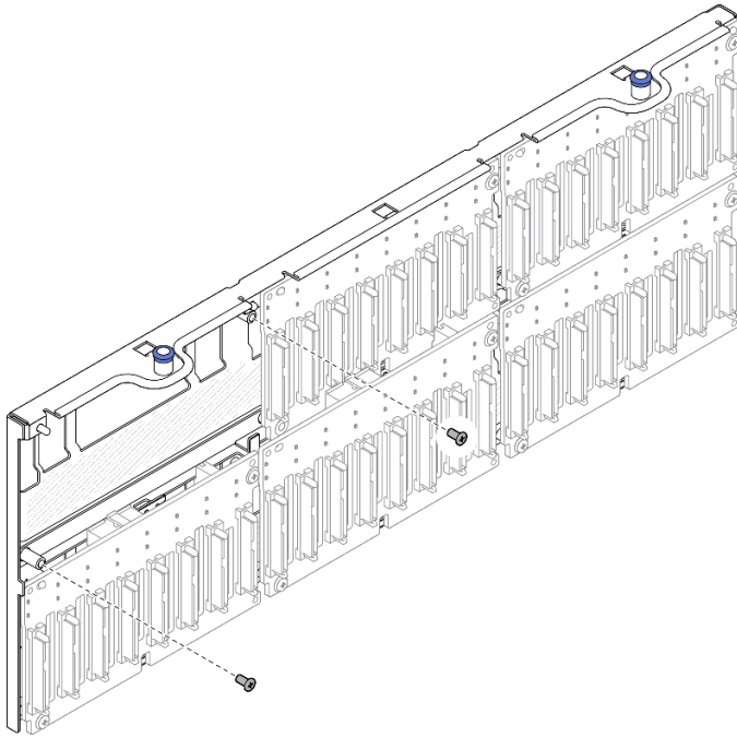
Figura 59. Tornillos de repuesto del transportador de la placa posterior
