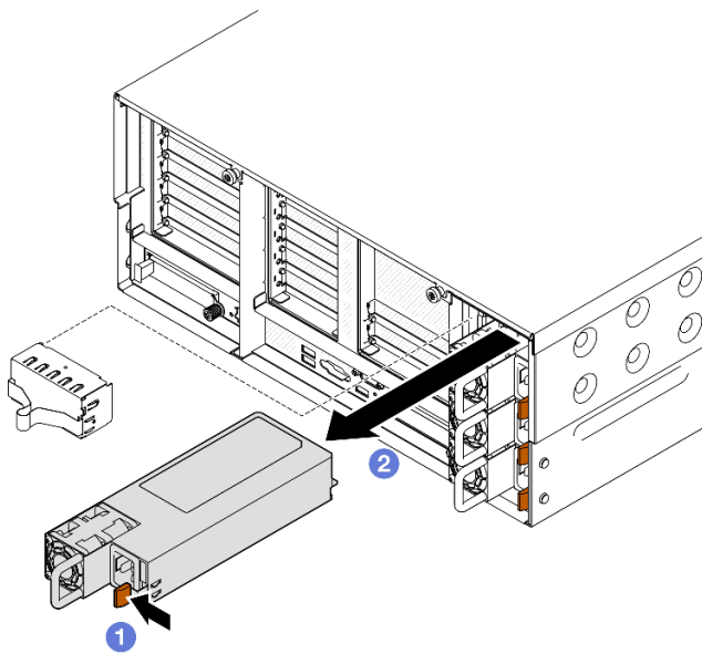
Figura 175. Extracción de la fuente de alimentación
