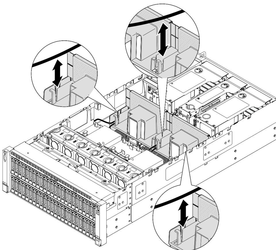
Figura 35. Levantamiento del cable para sacarlo del deflector de aire posterior
