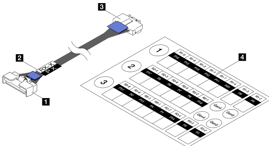
Figura 148. Cable de expansión PCIe
