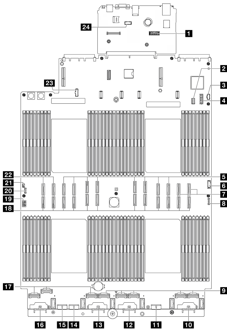
Figura 210. Conectores del conjunto de la placa del sistema
