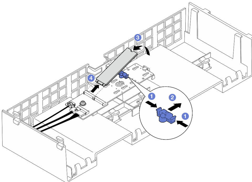
Figura 88. Extracción de la unidad M.2
