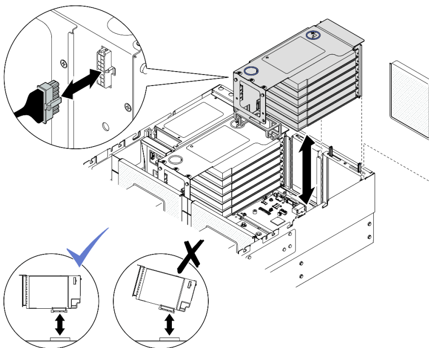
Figura 121. Instalación de la expansión de PCIe 1
