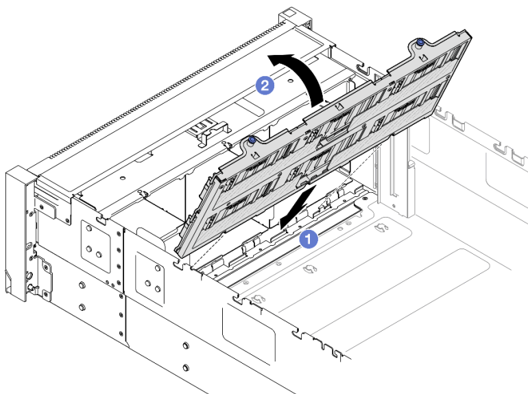
Figura 63. Instalación del conjunto del transportador de la placa posterior de la unidad
