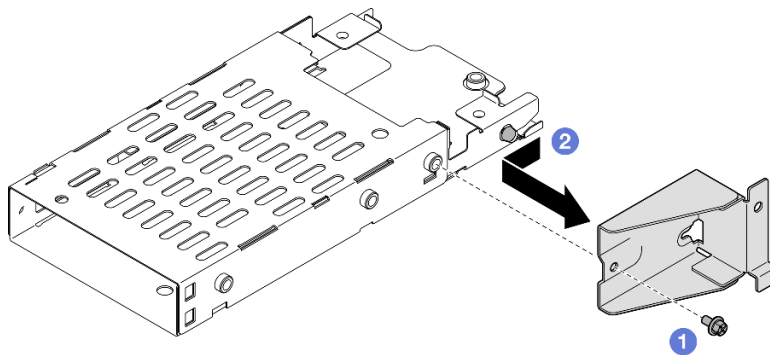
Figura 5. Extracción de la abrazadera del compartimento de la unidad de 7 mm
