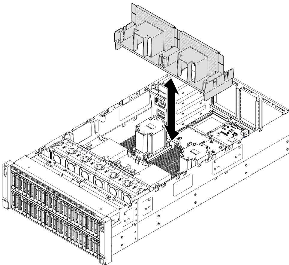
Figura 36. Extracción del deflector de aire posterior para PHM estándar de 3U
