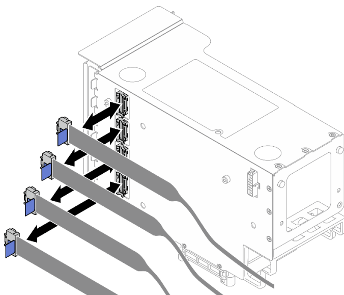
Figura 127. Desconexión de los cables de PCIe del exterior de la expansión
