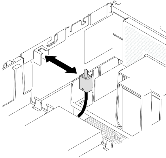
Figura 85. Extracción del conmutador de intrusión
