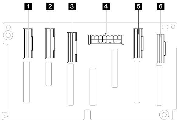
Figura 207. Conectores de la placa posterior de la unidad AnyBay de 8 bahías de 2,5"
