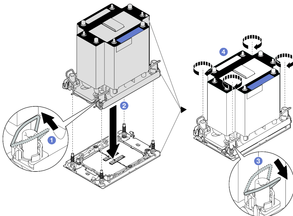
Figura 186. Instalación de un PHM estándar de 3U
