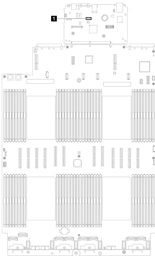
Figura 188. Desconexión del módulo de puerto serie
