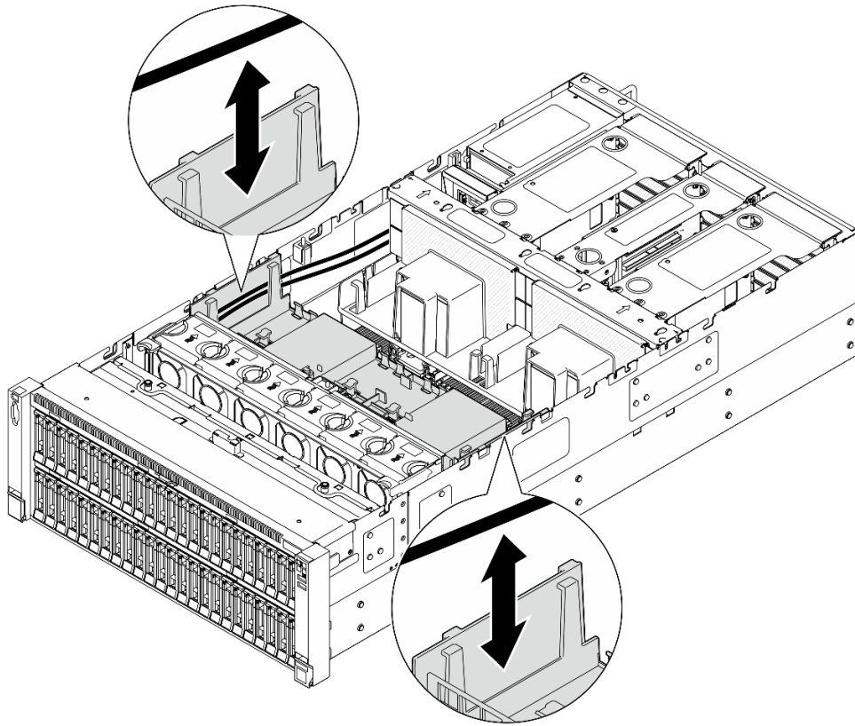
Figura 25. Levantamiento del cable para sacarlo del deflector de aire frontal
