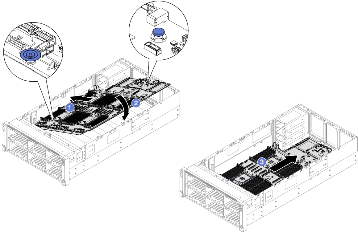
Figura 200. Instalación del conjunto de la placa del sistema
