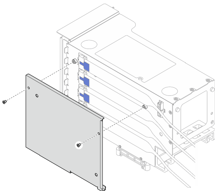
Figura 126. Extracción de la cubierta de la expansión
