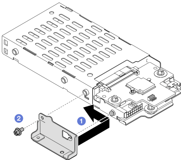
Figura 18. Instalación de la abrazadera del compartimiento de la unidad de 7 mm
