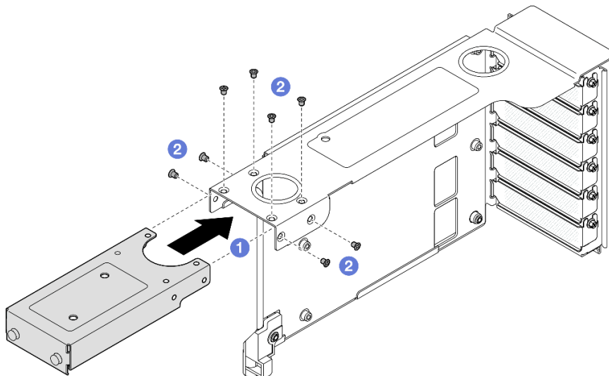
Figura 161. Instalación del amplificador de expansión de PCIe en expansión FH de PCIe
