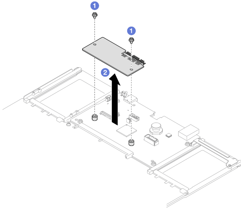
Figura 195. Extracción del firmware y módulo de seguridad de RoT
