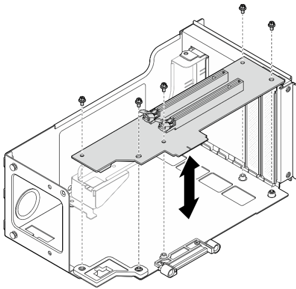
Figura 138. Instalación de la tarjeta de expansión PCIe a la expansión
