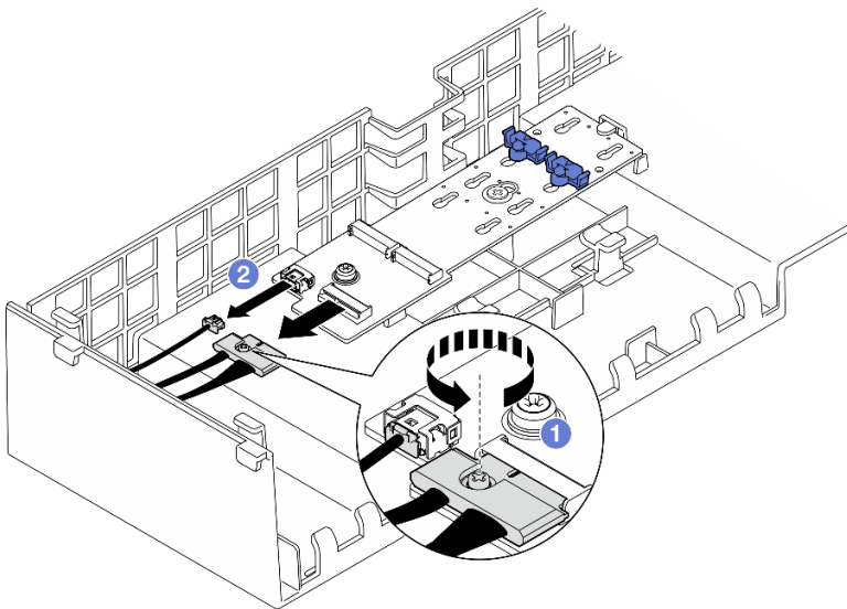
Figura 24. Desconexión del cable del adaptador de arranque M.2 SATA/NVMe o NVMe
