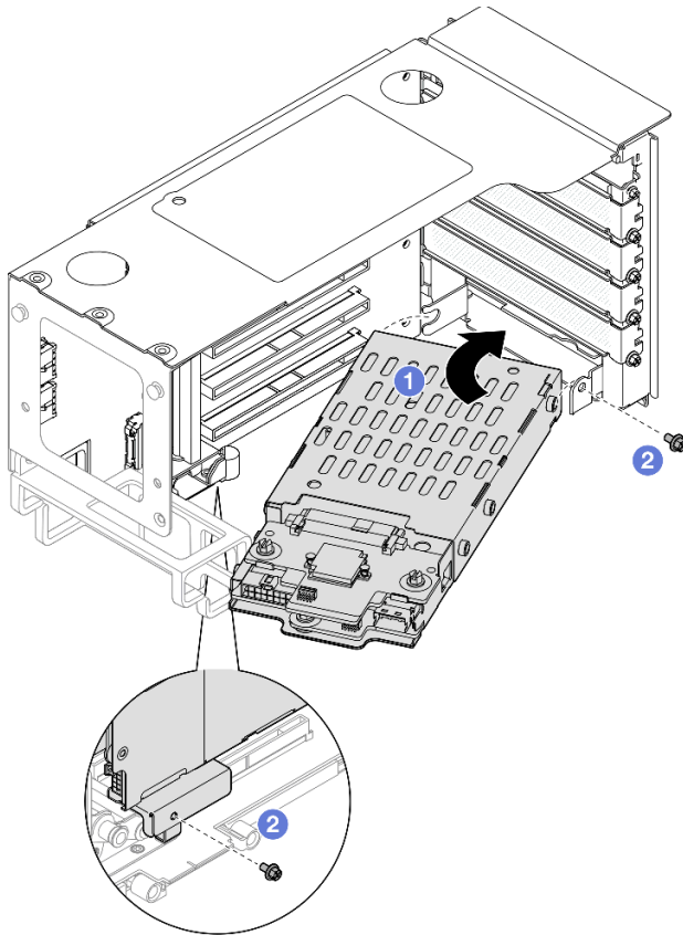
Figura 19. Instalación del compartimiento de la unidad de 7 mm en la expansión
