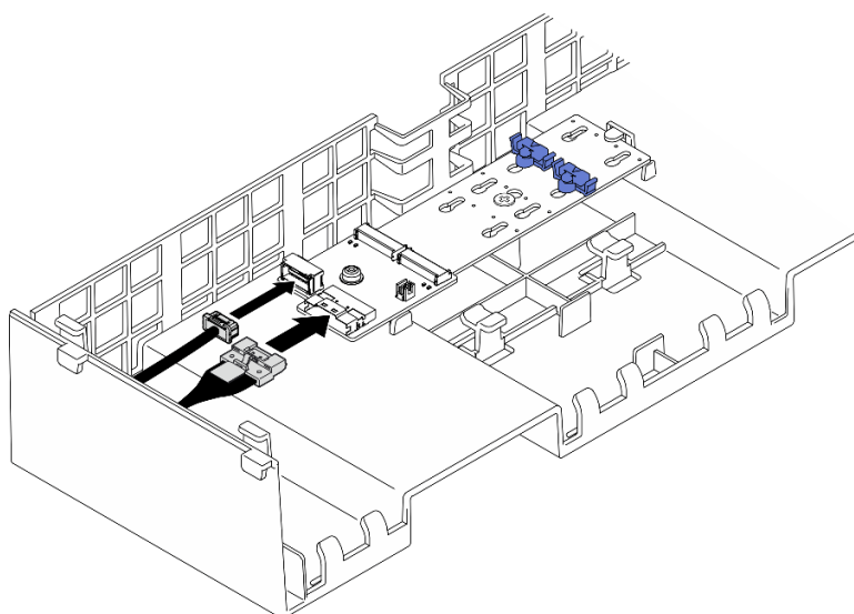
Figura 29. Conexión del cable al adaptador de arranque M.2 SATA/x4 NVMe
