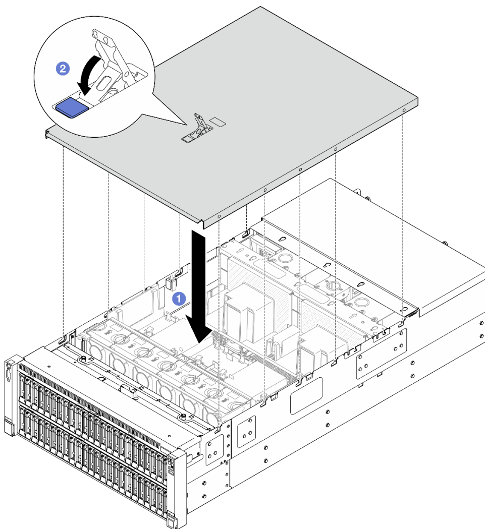
Figura 205. Instalación de la cubierta superior frontal
