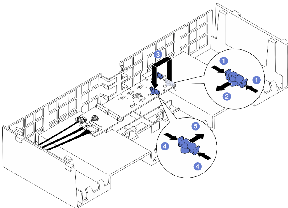
Figura 95. Ajuste del elemento de sujeción M.2
