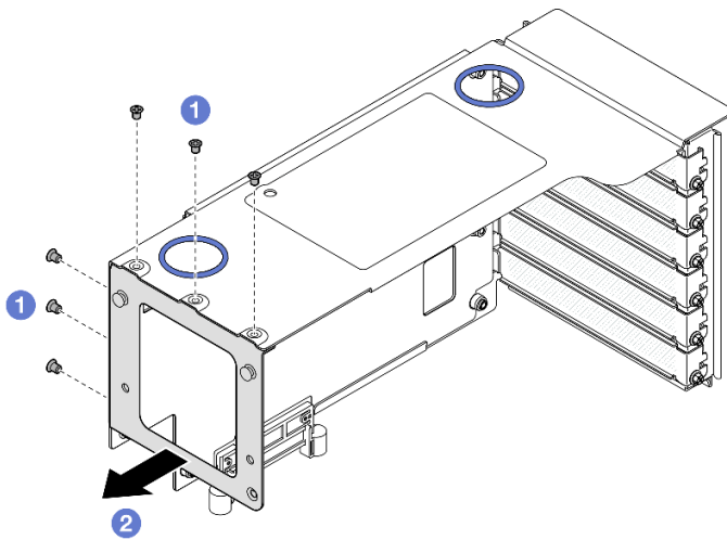
Figura 158. Extracción del relleno de la expansión FH de PCIe
