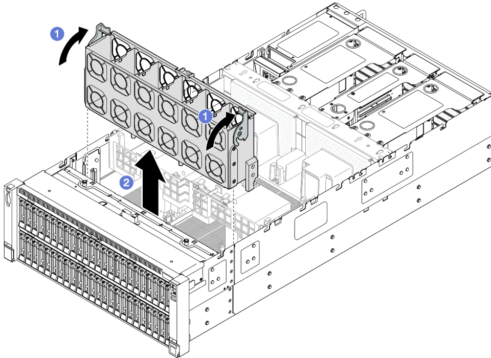
Figura 65. Extracción del compartimiento del ventilador
