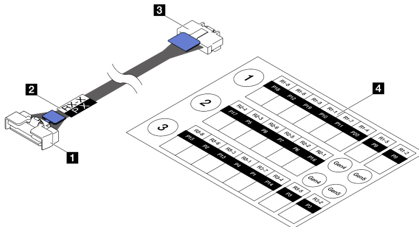
Figura 139. Cable de expansión PCIe
