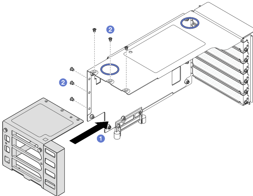
Figura 159. Instalación del ampliador de expansión de PCIe en expansión FH de PCIe
