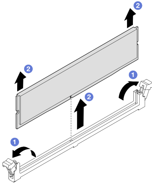
Figura 100. Extracción del módulo de memoria
