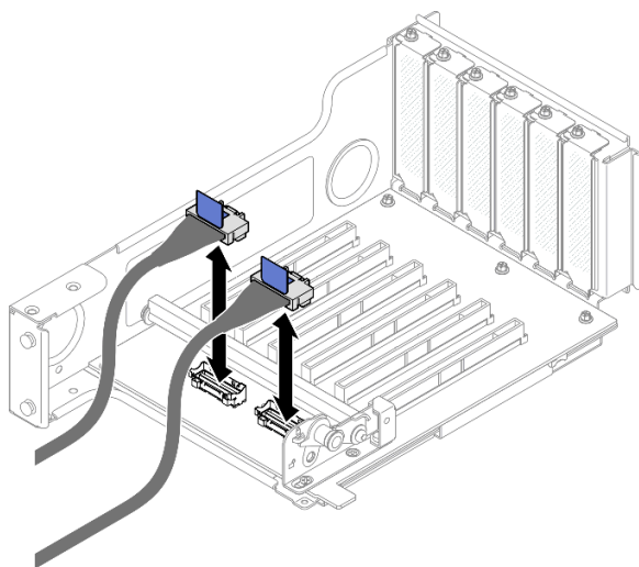
Figura 134. Desconexión de los cables de PCIe del interior de la expansión
