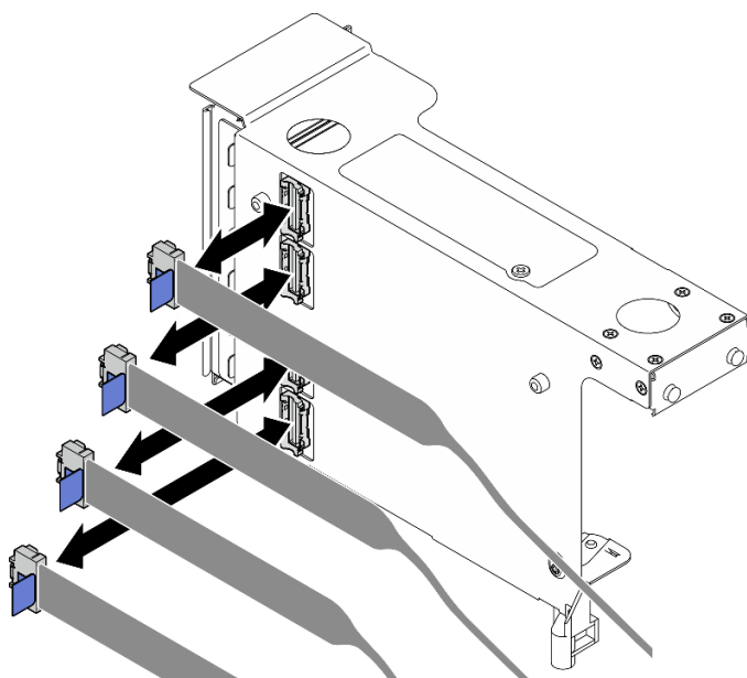
Figura 154. Conexión de los cables de la expansión de PCIe al exterior de la expansión
