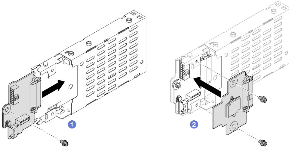
Figura 17. Instalación de la placa posterior de la unidad de 7 mm
