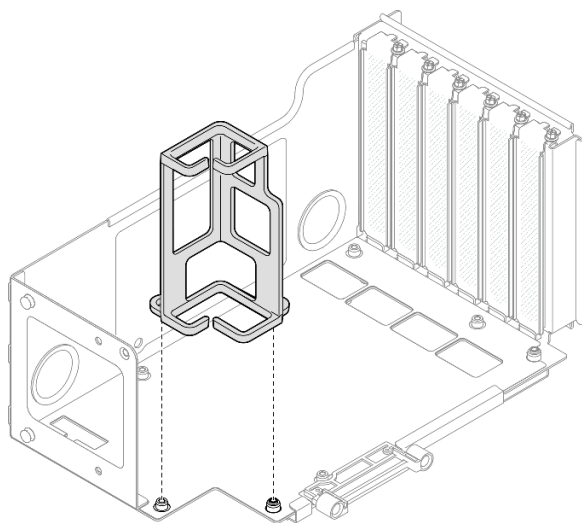
Figura 131. Extracción del soporte de cable de la expansión
