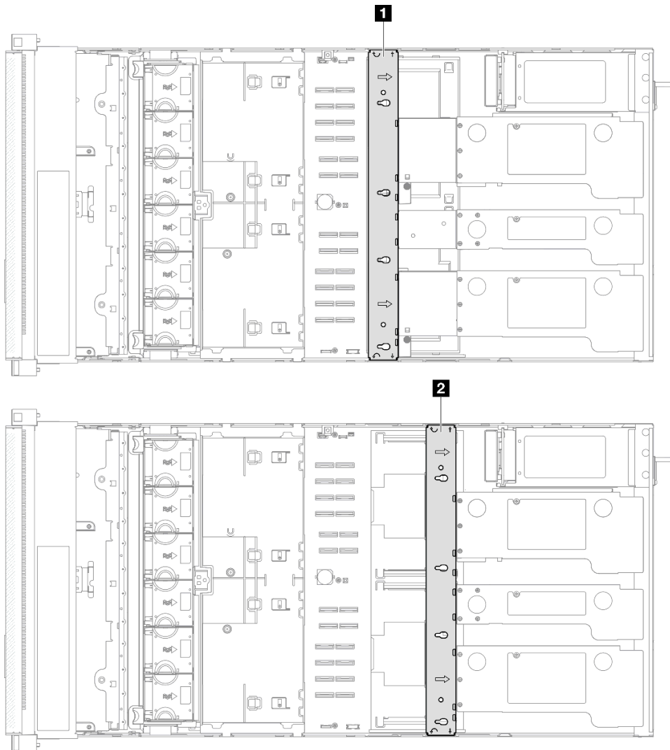
Figura 49. Ubicación de la barra cruzada
