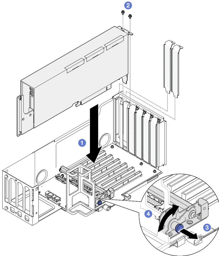
Figura 79. Instalación de un adaptador GPU en la expansión de PCIe
