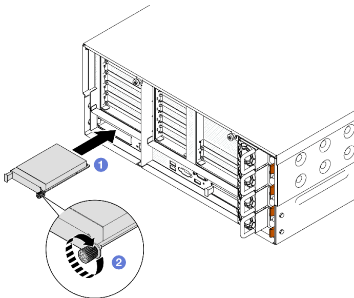
Figura 105. Instalación del módulo OCP
