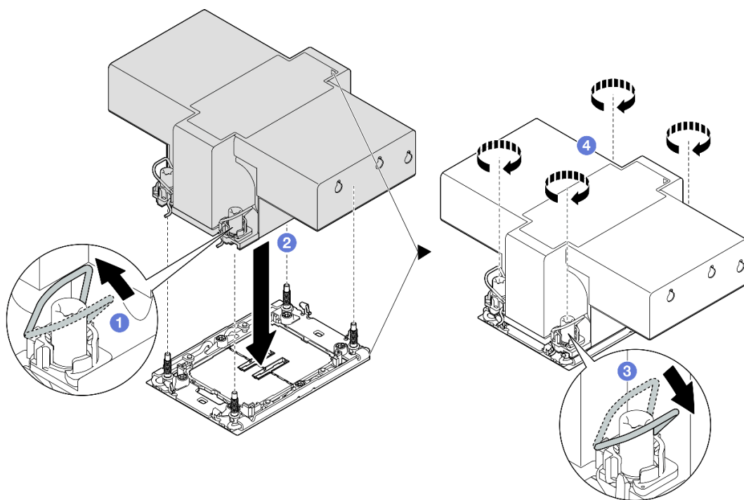
Figura 187. Instalación de un PHM de rendimiento de 2U
