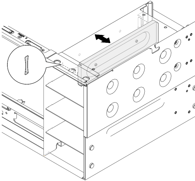
Figura 168. Extracción de soporte de fuente de alimentación
