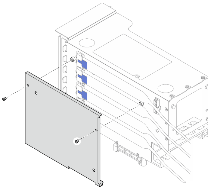
Figura 147. Instalación de la cubierta en la expansión
