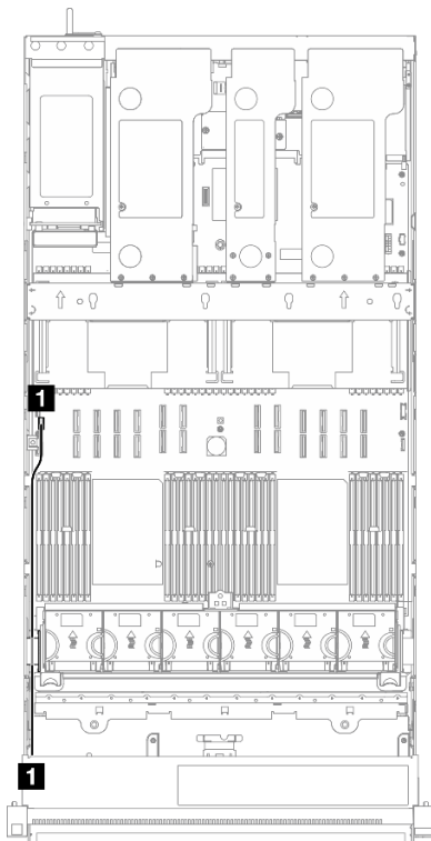
Figura 212. Disposición de los cables para el conector del auricular de diagnósticos externo
