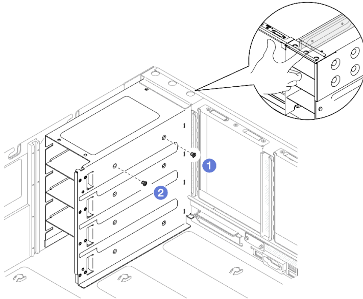
Figura 170. Fijación de soporte de fuente de alimentación
