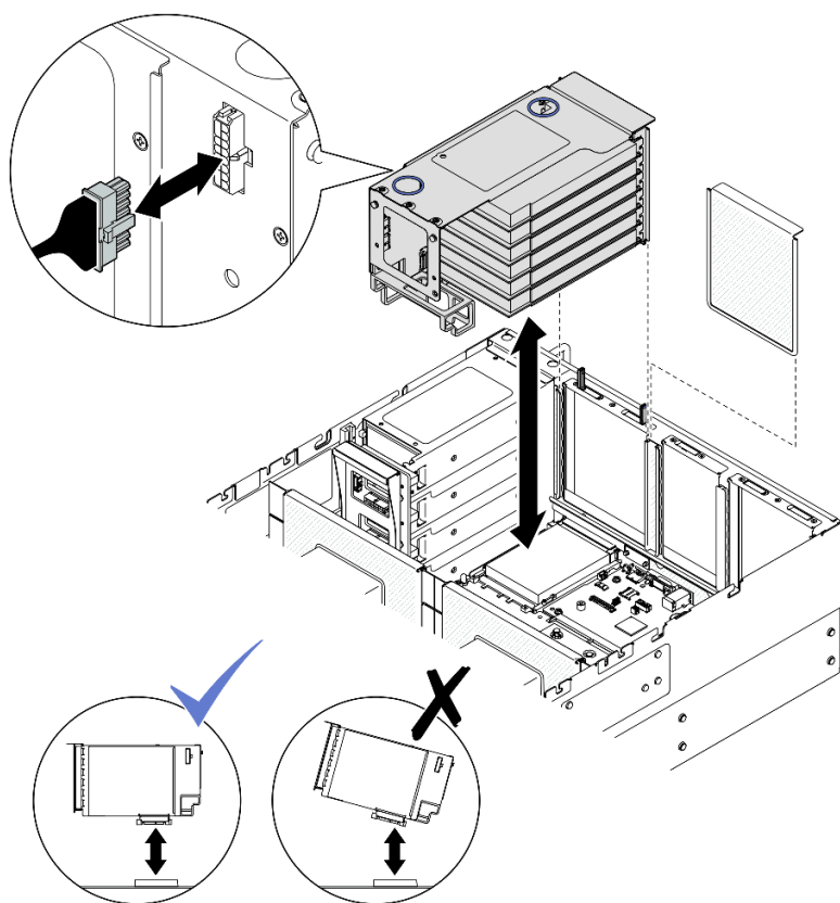
Figura 111. Extracción de la expansión de PCIe 3
