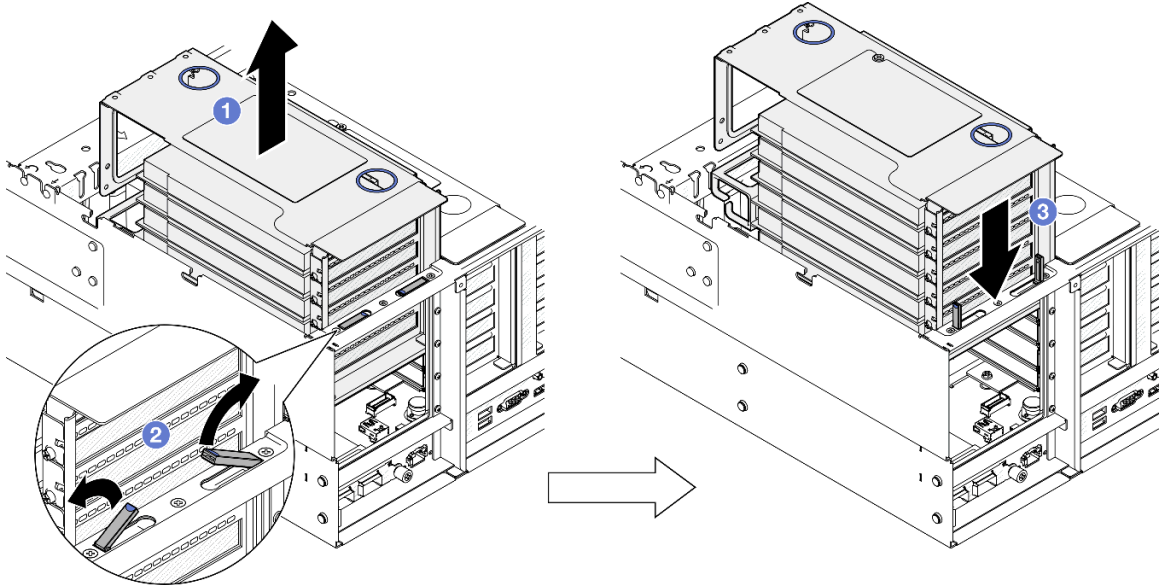
Figura 50. Desenganche de la expansión de PCIe
