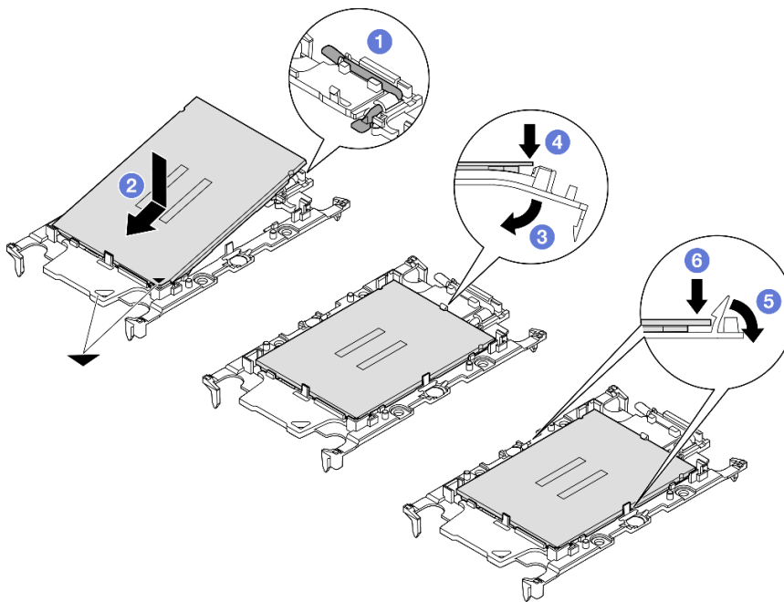
Figura 183. Instalación de un transportador de procesador
