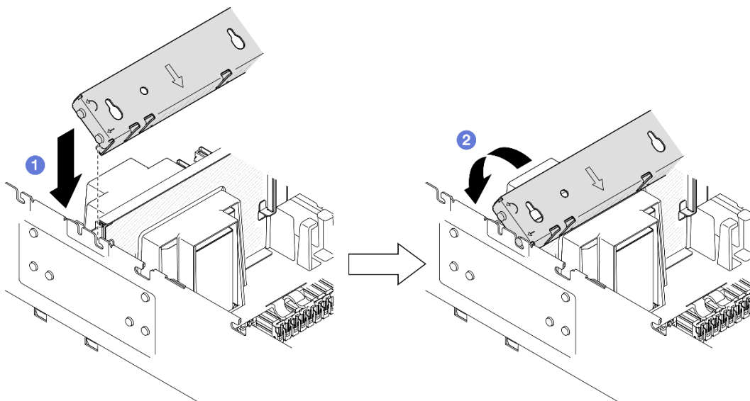
Figura 53. Instalación de la barra cruzada
