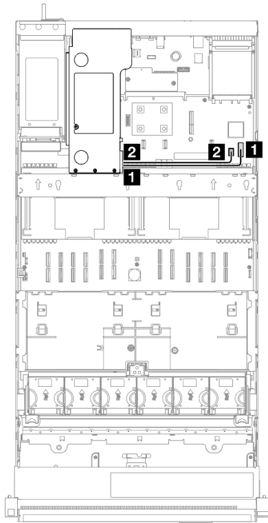
Figura 211. Disposición de los cables para la placa posterior de la unidad de 7 mm
