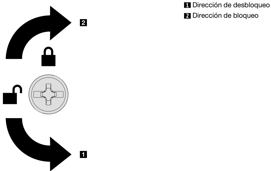
Figura 201. Dirección de bloqueo/desbloqueo de la cubierta superior frontal
