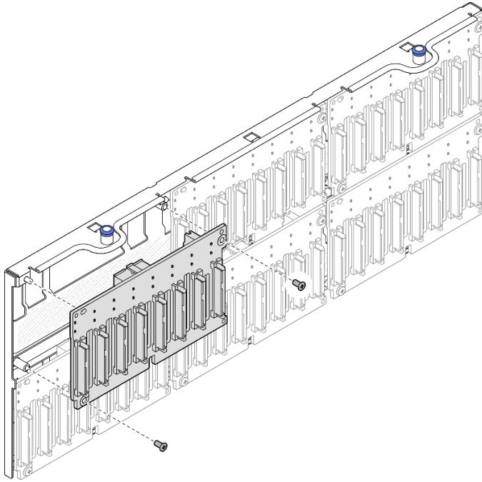
Figura 58. Extracción de la placa posterior del transportador
