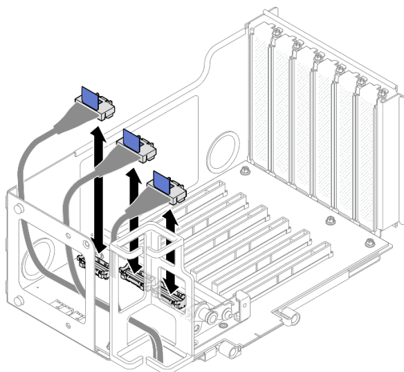
Figura 144. Conexión de los cables de la expansión de PCIe al interior de la expansión
