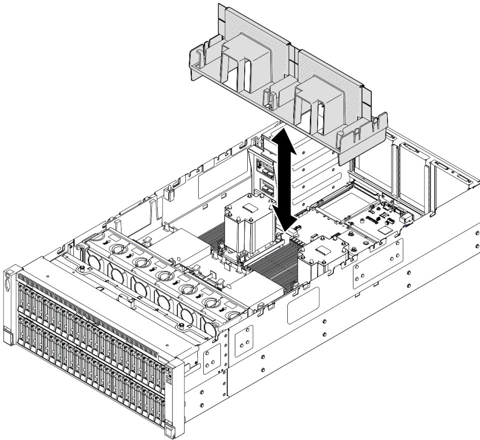
Figura 38. Instalación del deflector de aire posterior para PHM estándar de 3U
