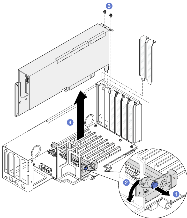
Figura 76. Extracción del adaptador GPU de la expansión de PCIe
