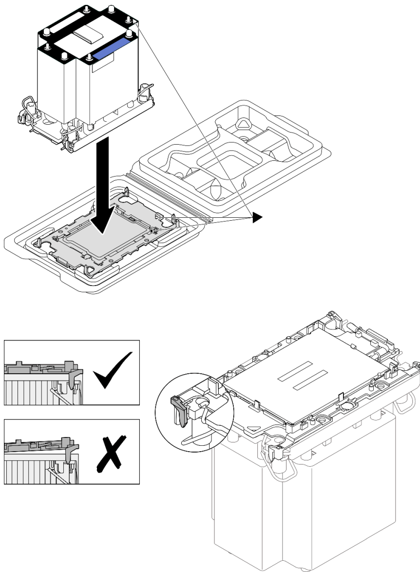
Figura 185. Ensamblaje del PHM con el procesador en la bandeja de envío
