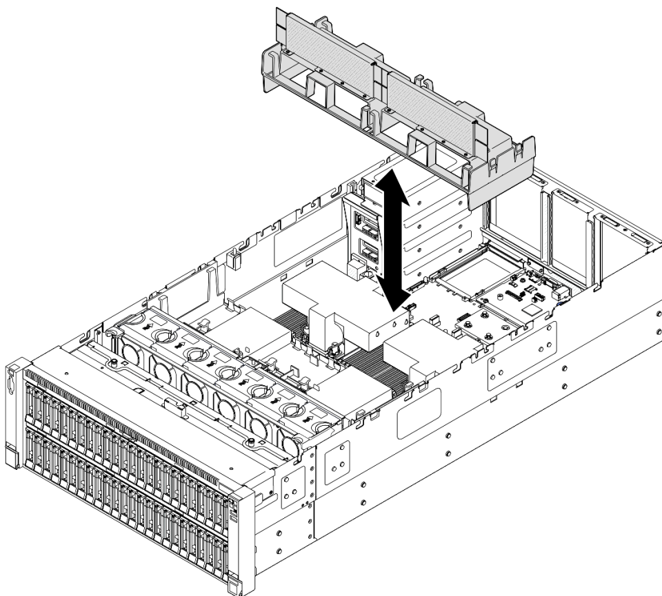
Figura 37. Extracción del deflector de aire posterior para PHM de rendimiento de 2U
