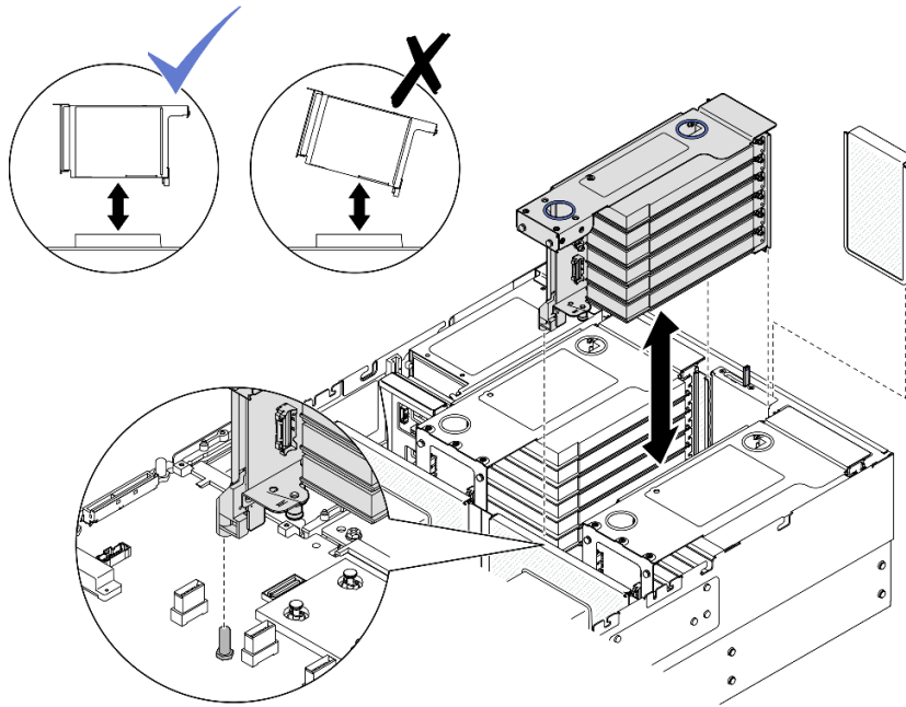
Figura 120. Instalación de la expansión de PCIe 2
